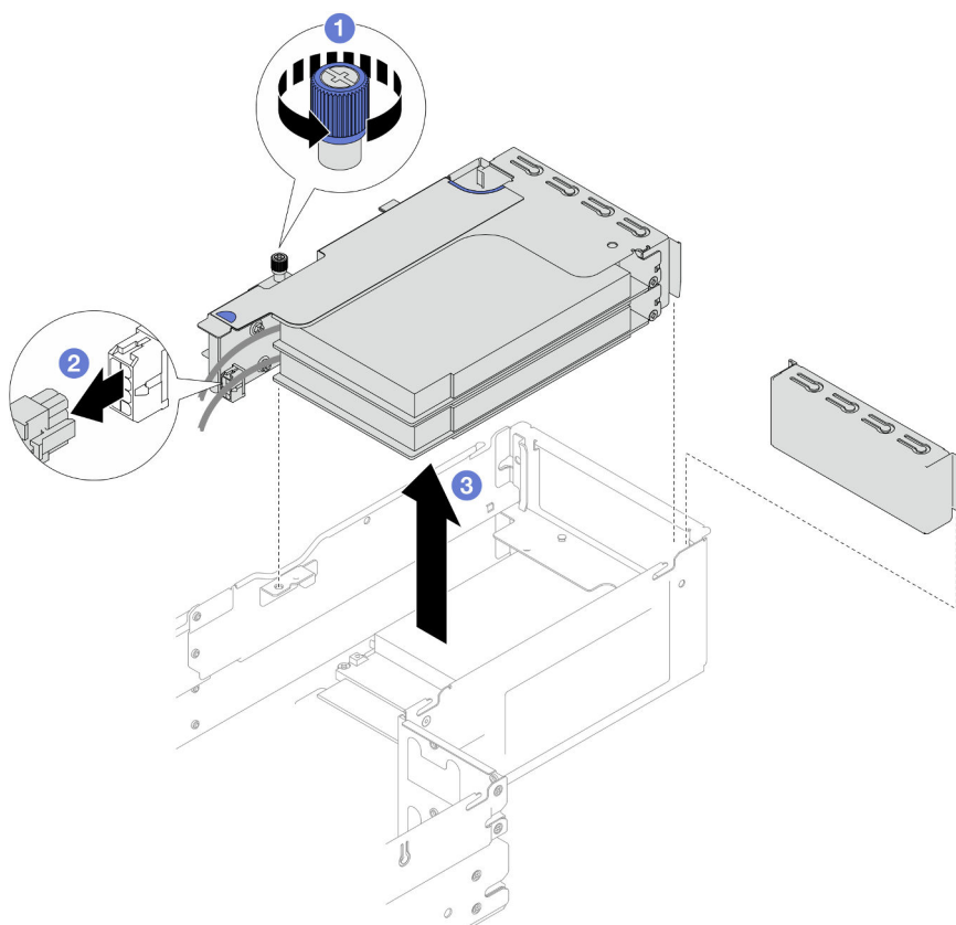
Figura 86. Remoção do conjunto de placa riser PCIe
