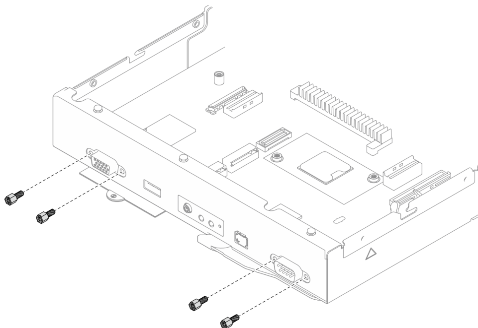
Figura 125. Instalação dos parafusos da placa-mãe na parte frontal
