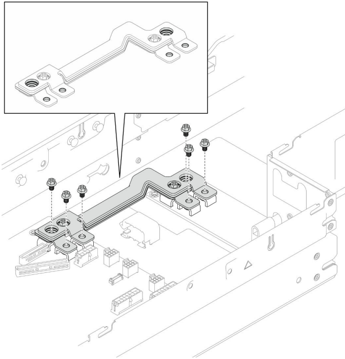
Figura 93. Remoção dos parafusos externos da barra do barramento de energia
