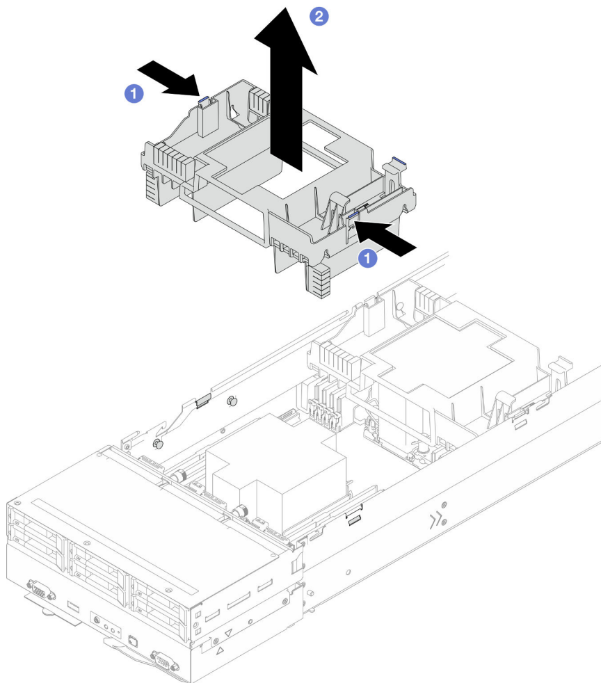
Figura 38. Remoção do defletor de ar frontal
