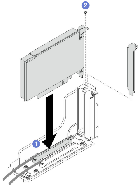
Figura 90. Instalação de um adaptador PCIe
