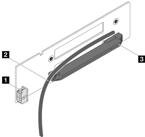
Figura 132. Conectores e cabos da placa riser PCIe de um slot
