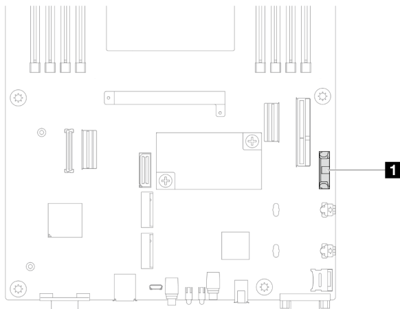
Figura 45. Local do soquete da bateria CMOS
