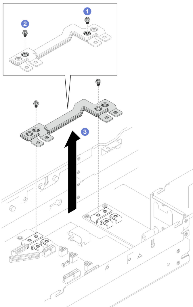
Figura 94. Remoção da barra de barramento de energia
