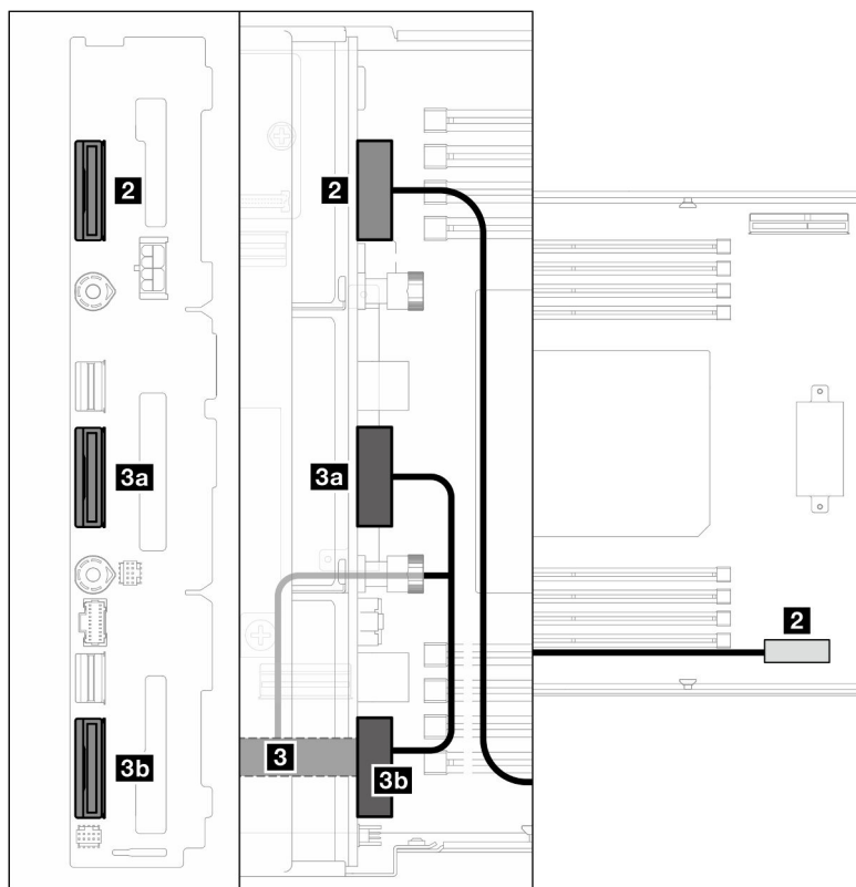
Figura 139. Roteamento de cabos NVMe
