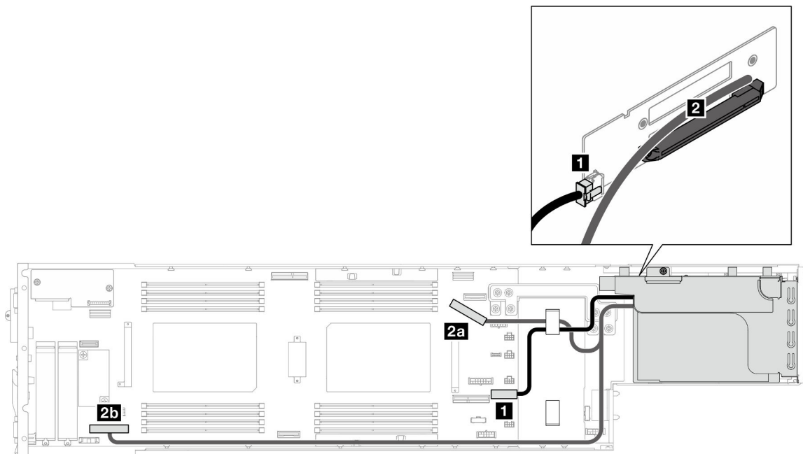
Figura 144. Roteamento de cabos da placa riser PCIe – um processador
