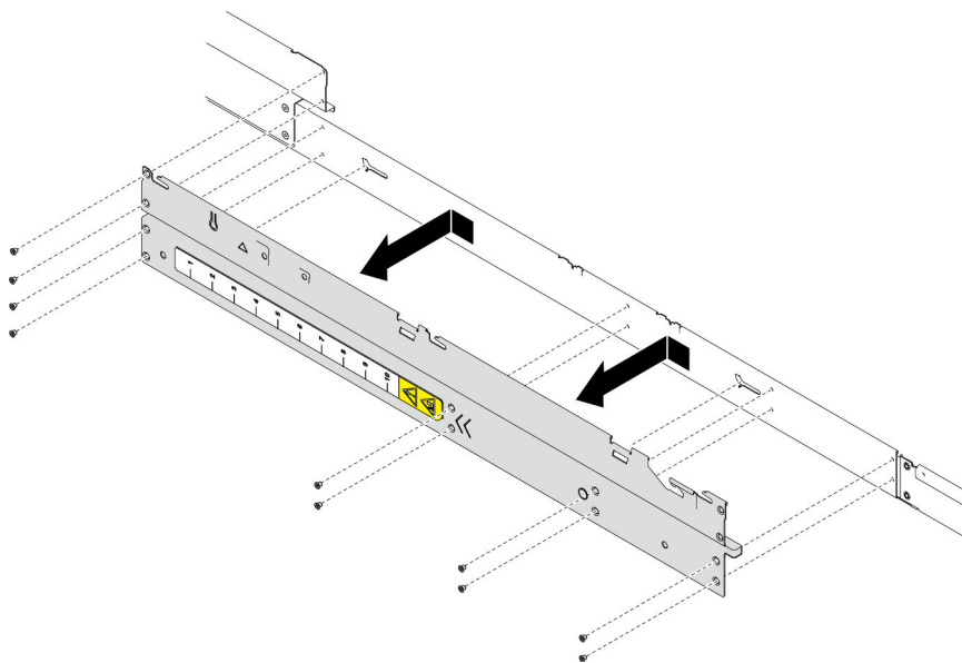
Figura 114. Remoção do suporte lateral
