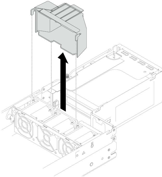
Figura 61. Remoção do duto de ar da GPU
