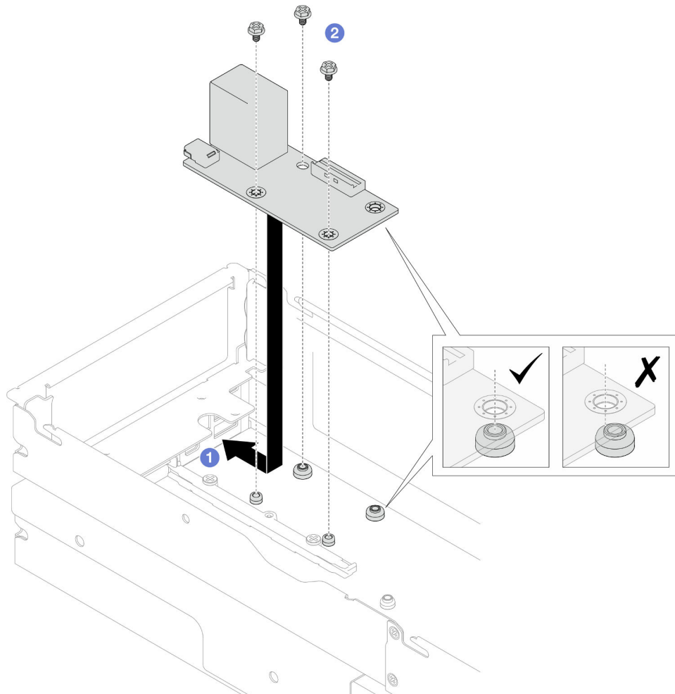
Figura 112. Instalação do módulo de E/S traseiro
