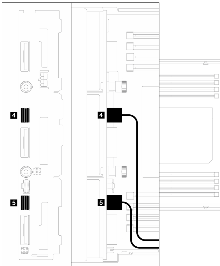
Figura 140. Cabos SATA no backplane da unidade
