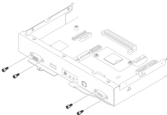
Figura 121. Remoção dos parafusos
