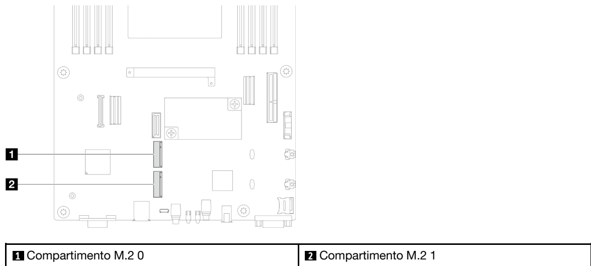
Figura 74. Local dos compartimentos M.2 na placa-mãe
