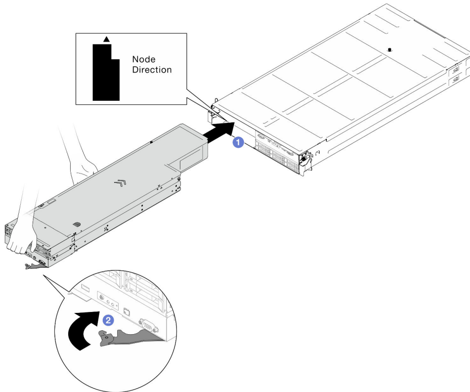
Figura 36. Instalação do nó na bandeja esquerda
