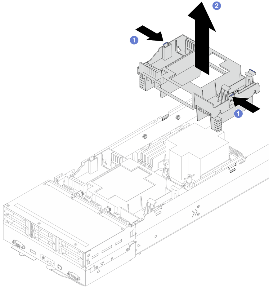
Figura 39. Remoção do defletor de ar traseiro
