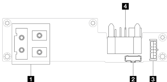
Figura 134. Conectores da placa de distribuição de energia
