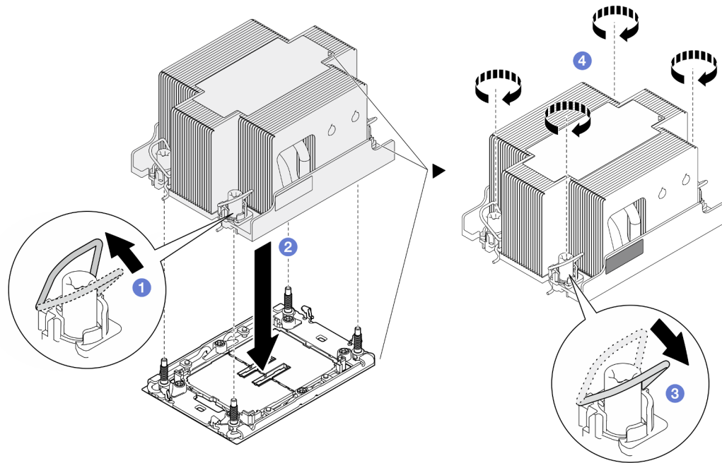
Figura 108. Instalação de um PHM padrão de 2U
