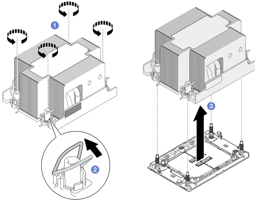
Figura 100. Remoção do PHM padrão de 2U
