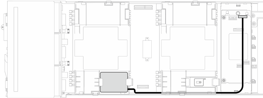
Figura 143. Cabo do módulo de energia flash e RAID CFF
