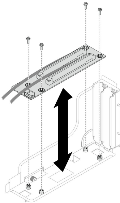
Figura 91. Substituição da placa riser PCIe
