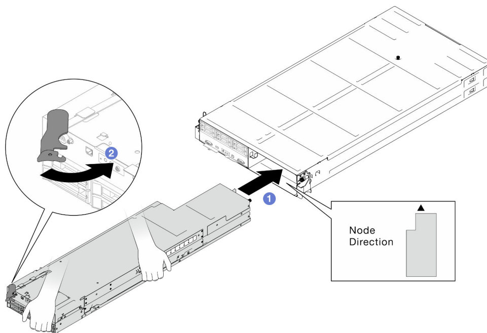
Figura 37. Instalação do nó na bandeja direita
