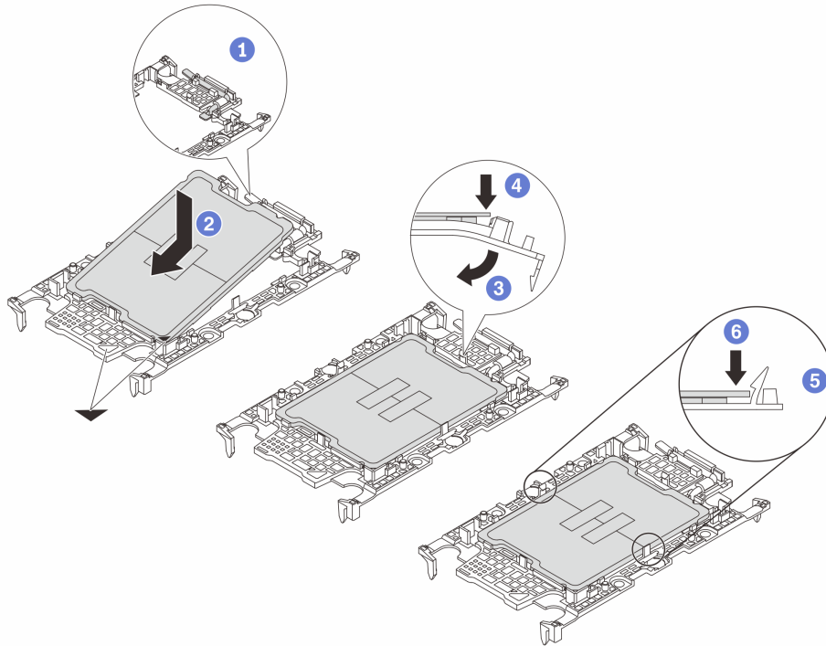
Figura 105. Instalação da portadora de processador
