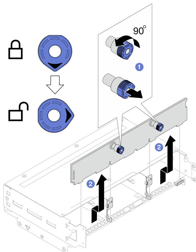
Figura 50. Remoção do backplane de unidade
