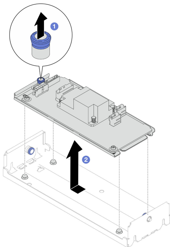
Figura 42. Remoção do adaptador CFF interno
