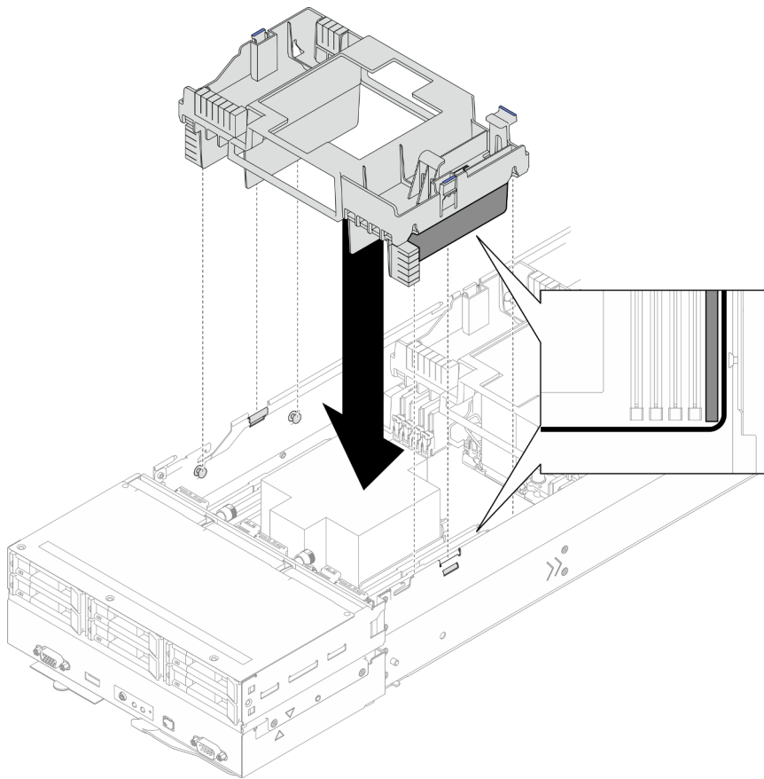
Figura 40. Instalação do defletor de ar frontal
