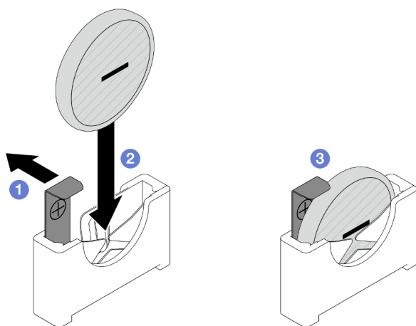
Figura 48. Instalação de uma bateria CMOS
