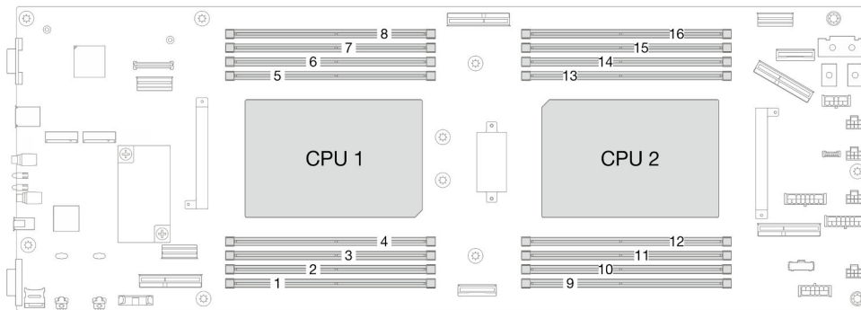
Figura 78. Layout de módulos de memória e processadores
