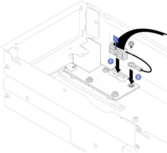
Figura 113. Instalação do cabo de E/S traseiro e do cabo de aterramento
