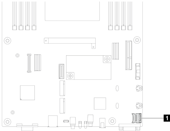
Figura 82. Local do soquete MicroSD
