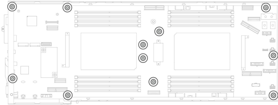
Figura 122. Remoção dos parafusos
