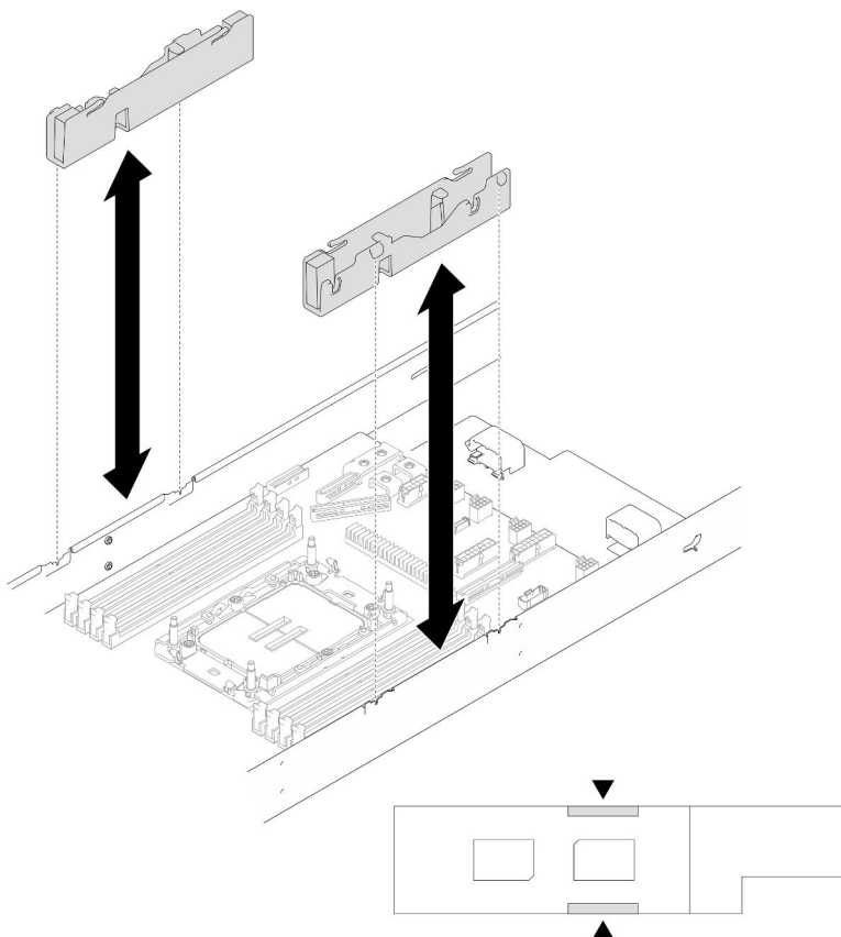
Figura 127. Substituição do duto de cabos
