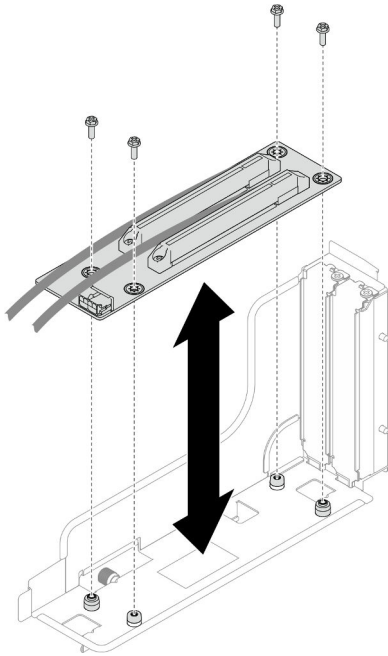
Figura 89. Substituição da placa riser PCIe
