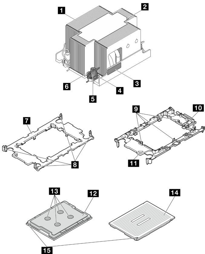
Figura 99. Componentes do PHM
