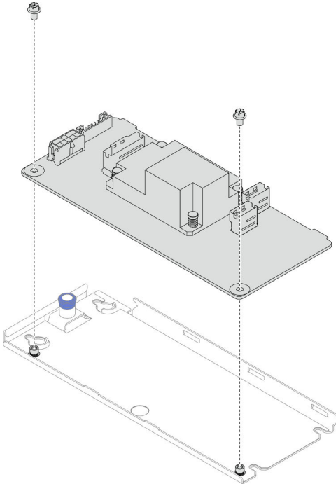
Figura 43. Separação do adaptador RAID CFF interno da bandeja
