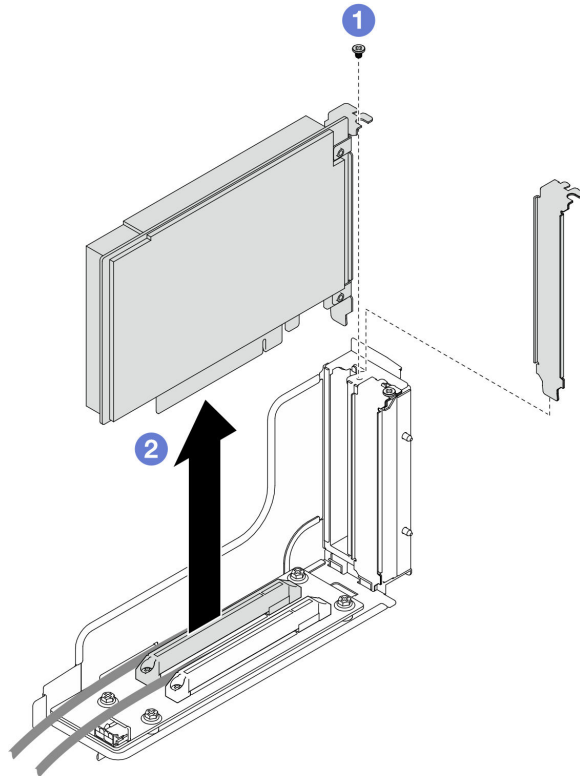
Figura 88. Remoção de um adaptador PCIe
