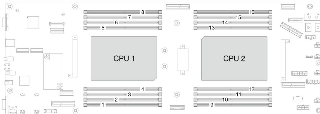
Figura 15. Layout de módulos de memória e processadores
