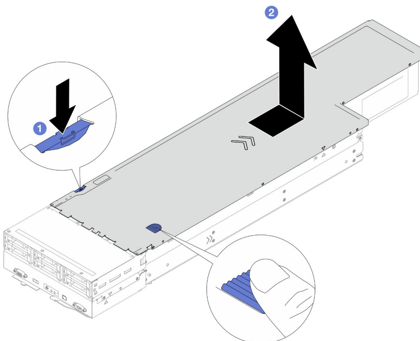
Figura 128. Remoção da tampa superior
