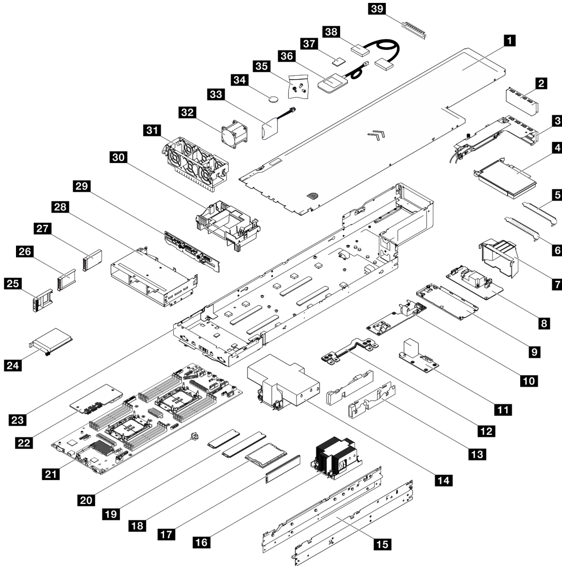
Figura 11. Componentes do nó
