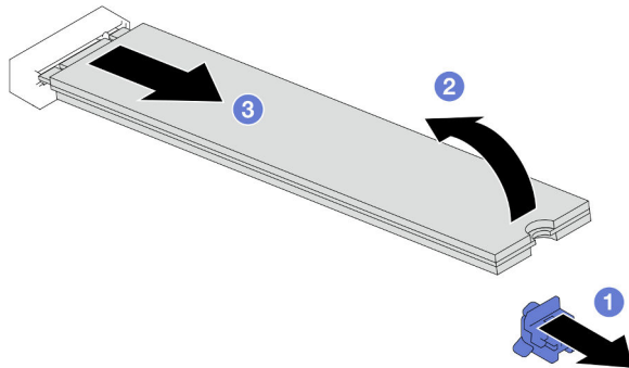
Figura 72. Remoção de uma unidade M.2
