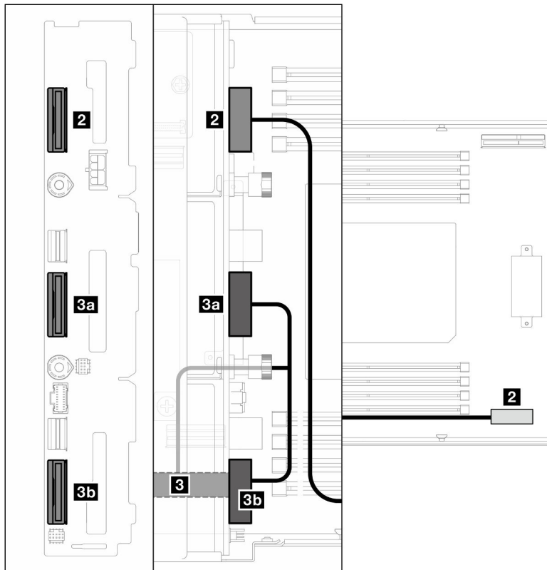
Figura 136. Roteamento de cabos NVMe
