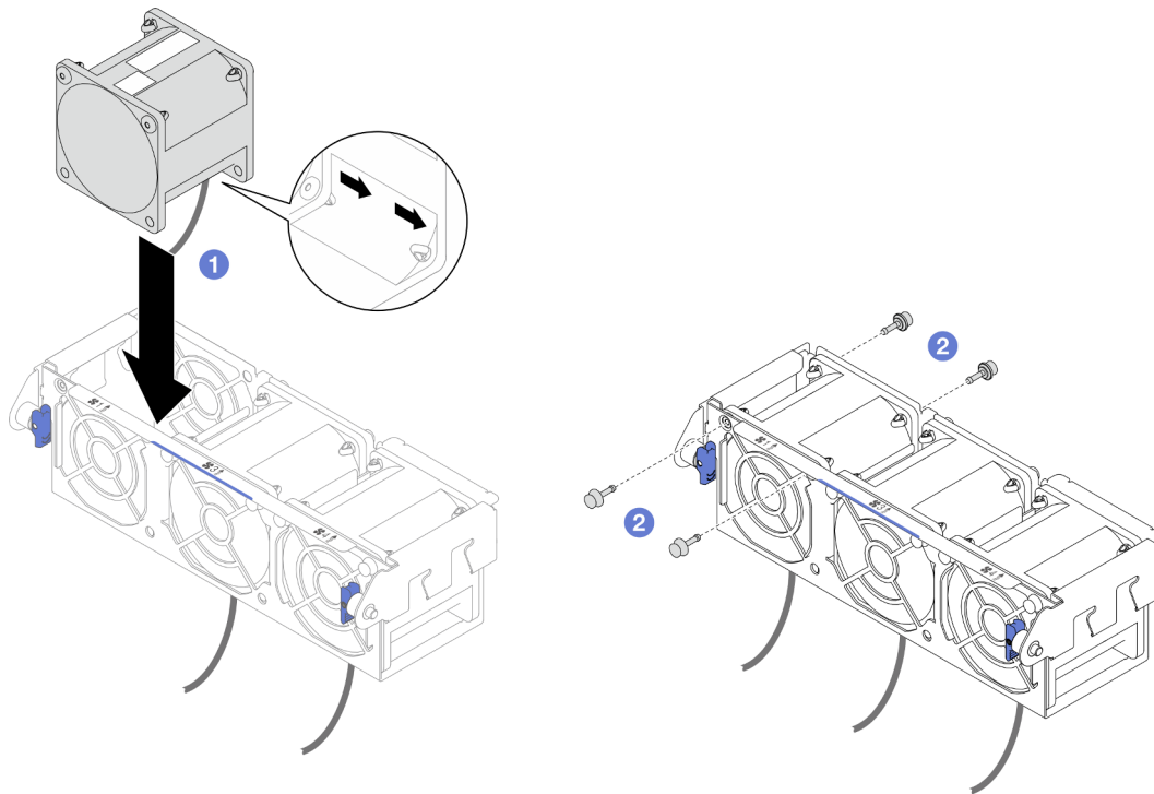
Figura 55. Instalação do ventilador
