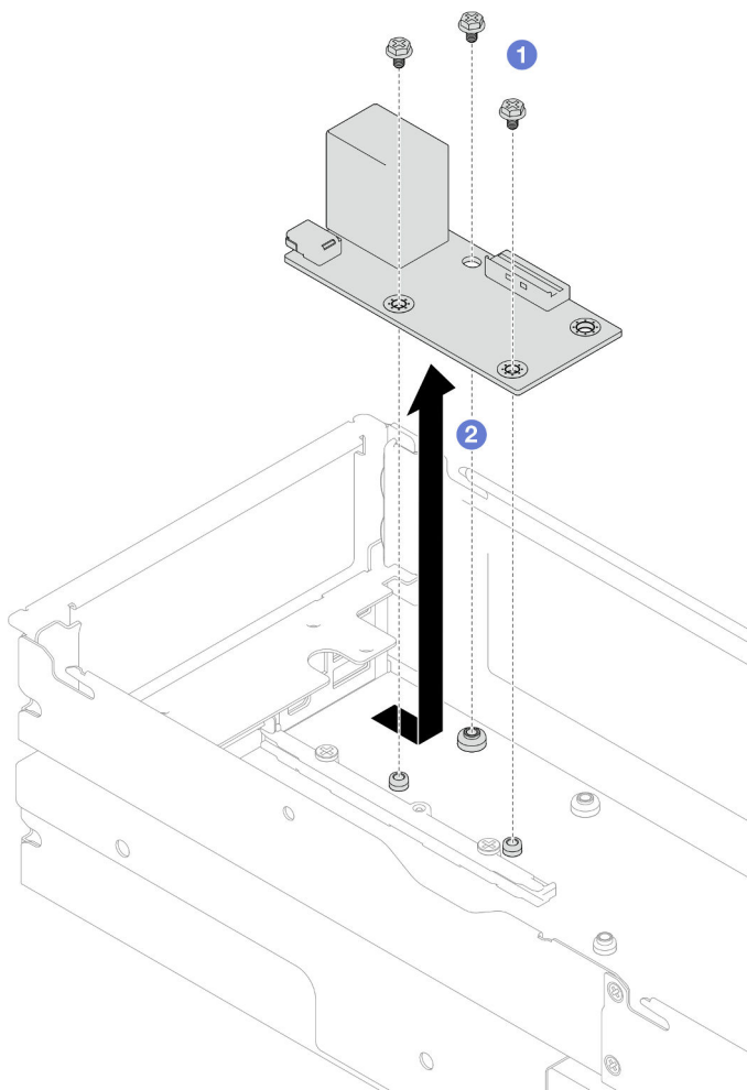
Figura 111. Remoção do módulo de E/S traseiro
