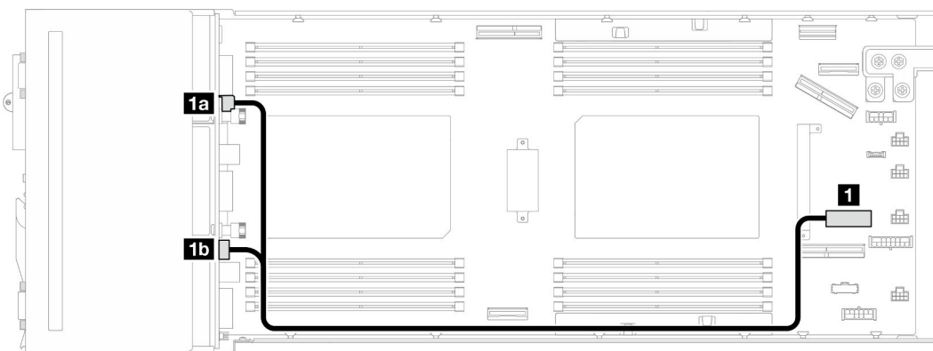
Figura 138. Roteamento de cabos de alimentação do backplane da unidade
