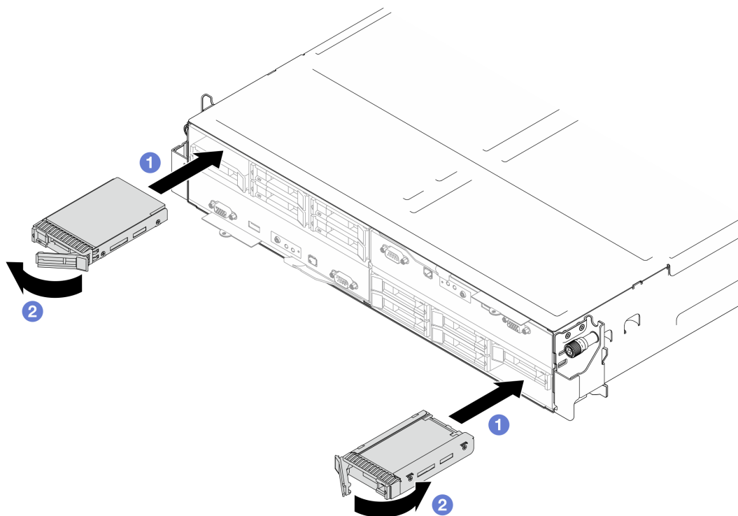
Figura 67. Instalação de uma unidade de estado sólido de 7 mm
