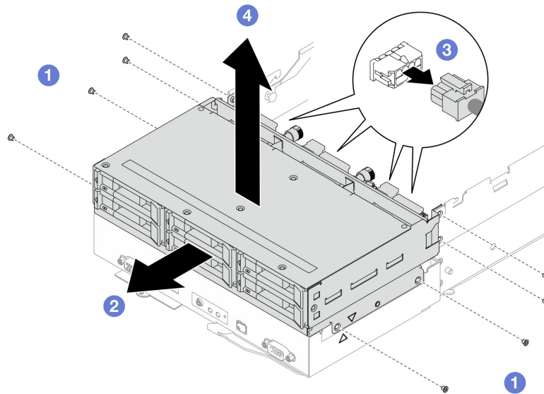
Figura 49. Remoção do conjunto da gaiola de unidade
