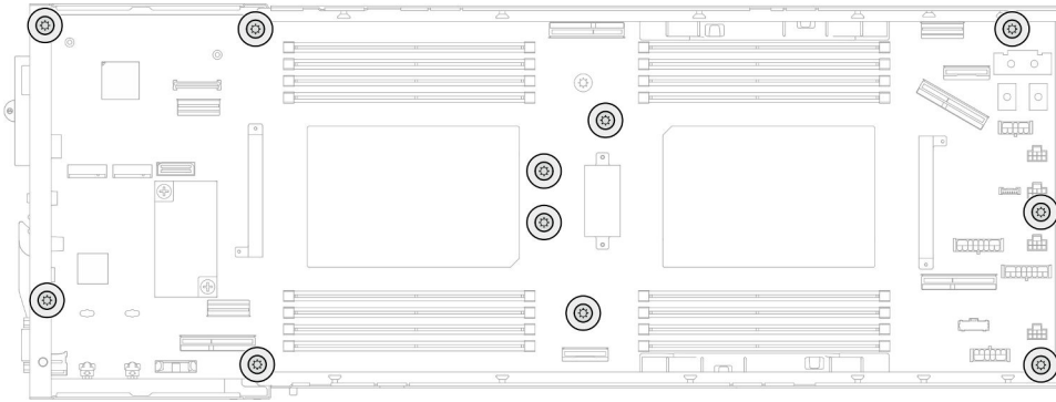
Figura 126. Instalação dos parafusos na placa-mãe
