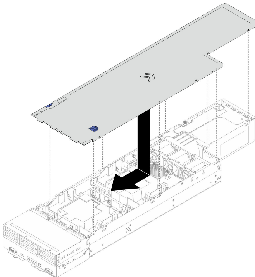
Figura 129. Instalação da tampa superior
