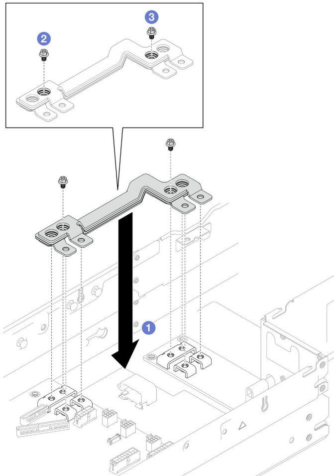
Figura 95. Instalação da barra de barramento de energia
