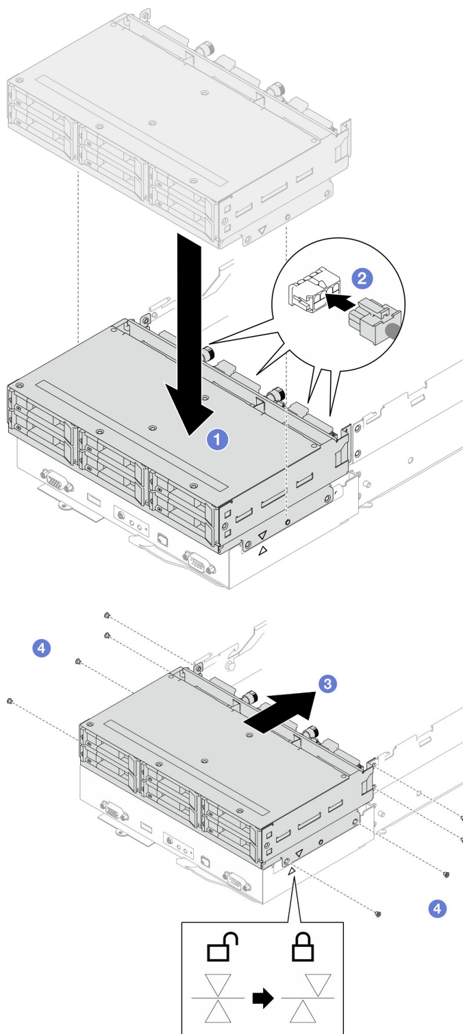
Figura 52. Instalação do conjunto da gaiola de unidade
