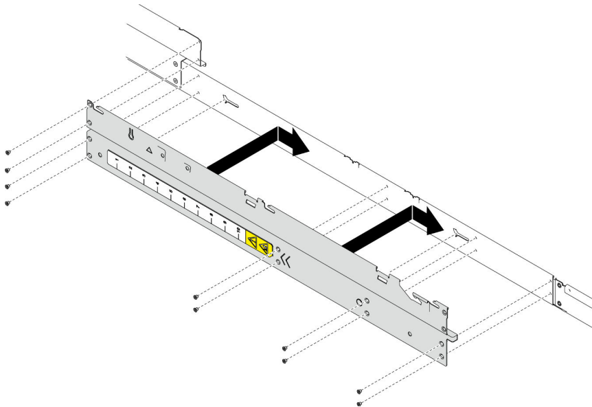
Figura 115. Instalação do suporte lateral
