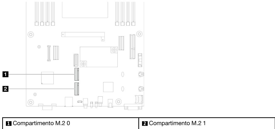
Figura 71. Local dos compartimentos M.2 na placa-mãe
