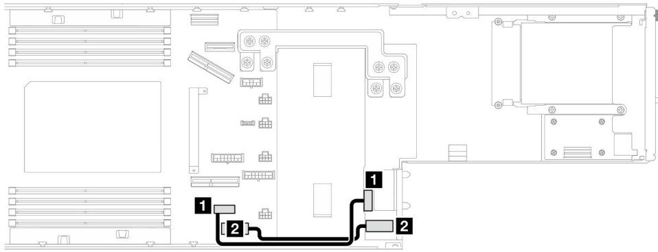
Figura 146. Roteamento de cabos da placa de distribuição de energia
