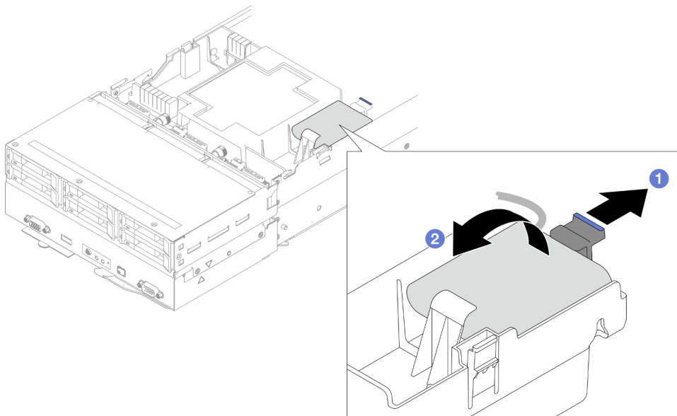
Figura 57. Remoção do módulo de energia flash
