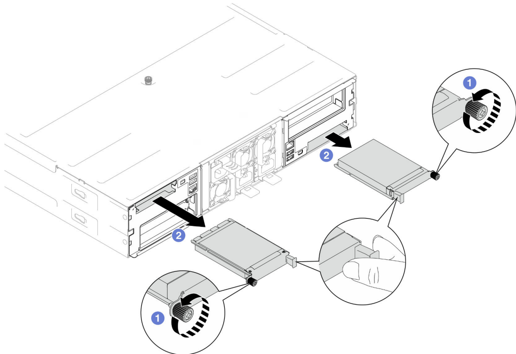
Figura 84. Remoção do módulo OCP traseiro
