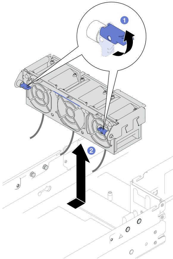
Figura 53. Remoção da gaiola do ventilador
