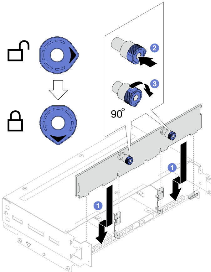
Figura 51. Instalação do backplane da unidade
