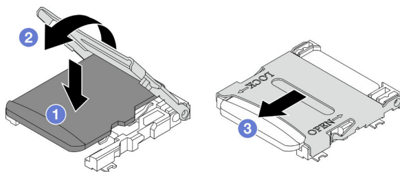
Figura 83. Instalação do cartão microSD
