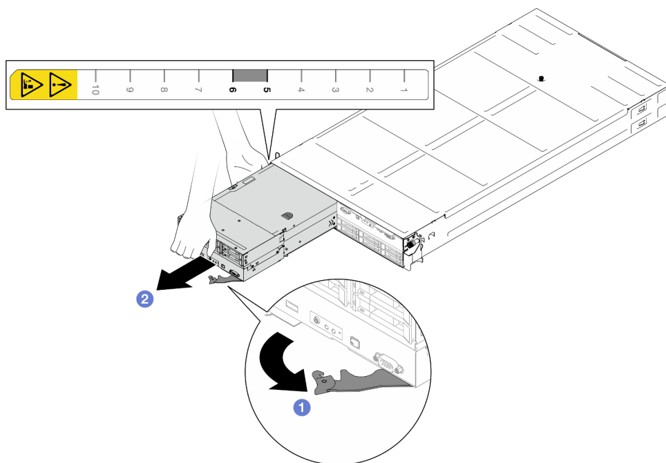
Figura 30. Remoção do nó da bandeja esquerda
