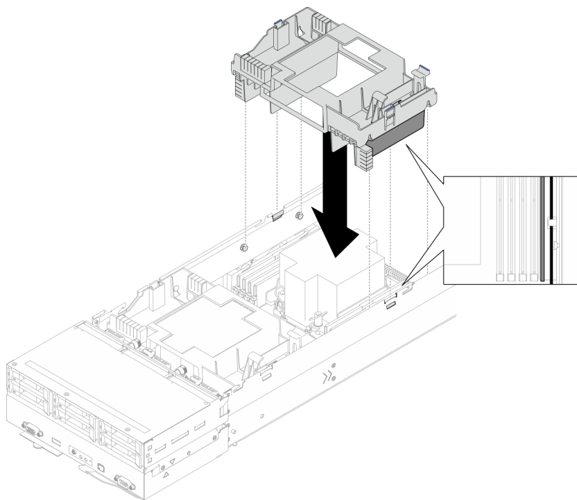
Figura 41. Instalação do defletor de ar traseiro
