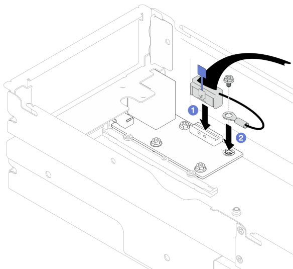
Figura 148. Instalação do cabo de E/S traseiro e do cabo de aterramento
