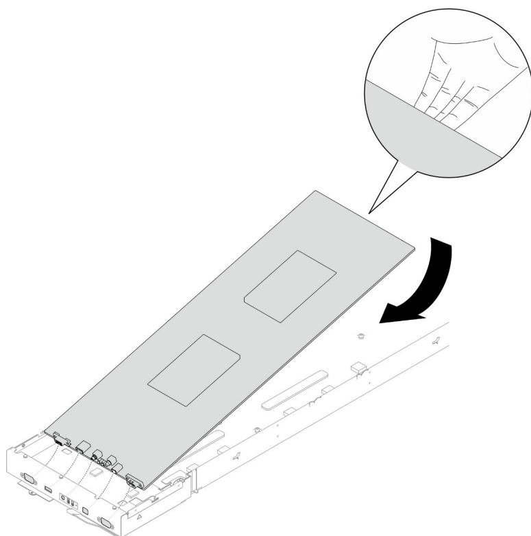
Figura 124. Instalação da placa-mãe
