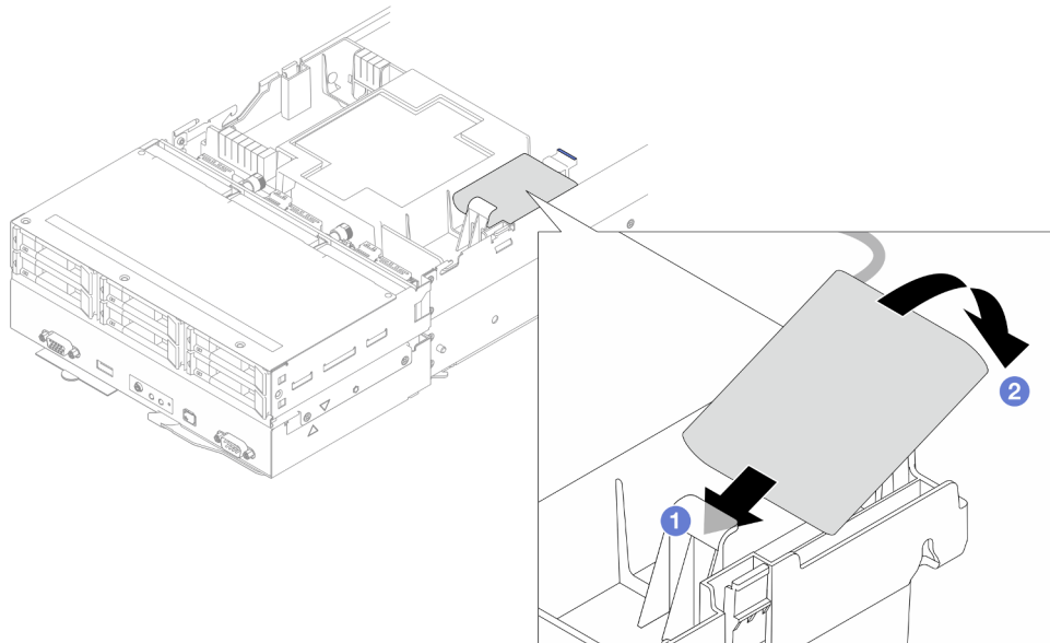
Figura 58. Instalação do módulo de energia flash
