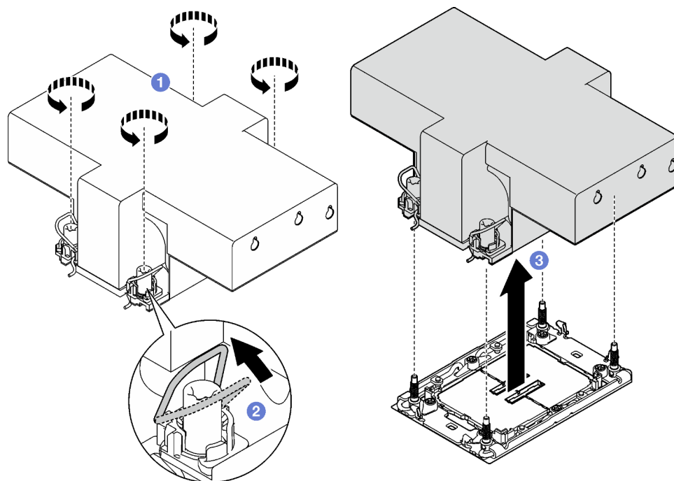
Figura 101. Remoção do PHM de desempenho 2U
