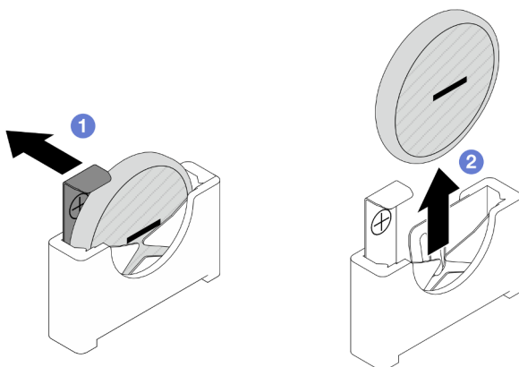
Figura 46. Remoção da bateria CMOS
