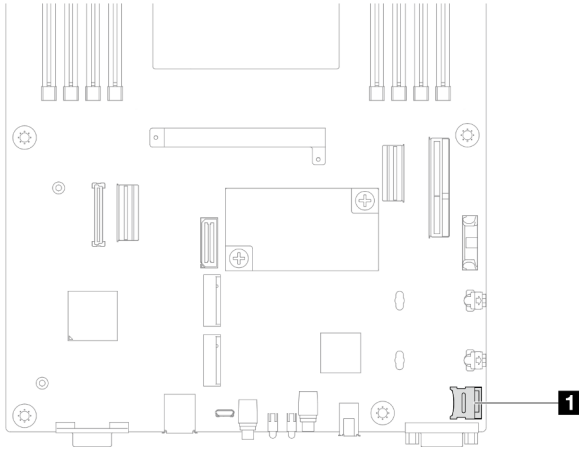
Figura 80. Local do soquete MicroSD
