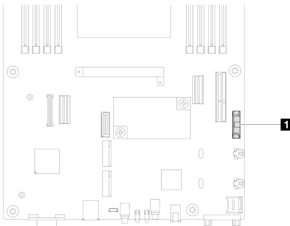
Figura 47. Local do soquete da bateria CMOS
