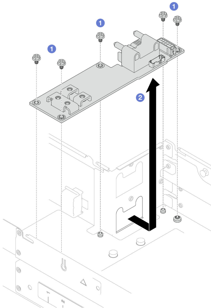
Figura 97. Remoção da placa de distribuição de energia
