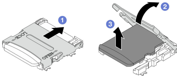
Figura 81. Remoção do cartão microSD
