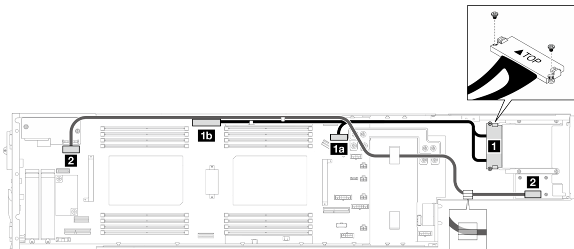
Figura 147. Cabos do módulo de E/S traseiro e do módulo OCP
