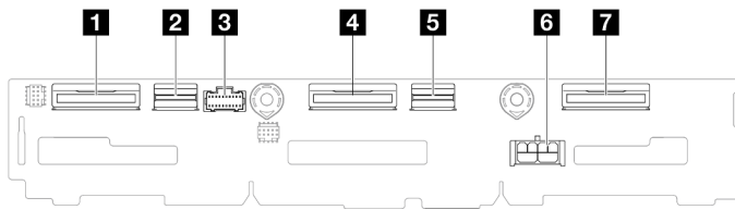
Figura 130. Backplane da unidade de 2,5 polegadas
