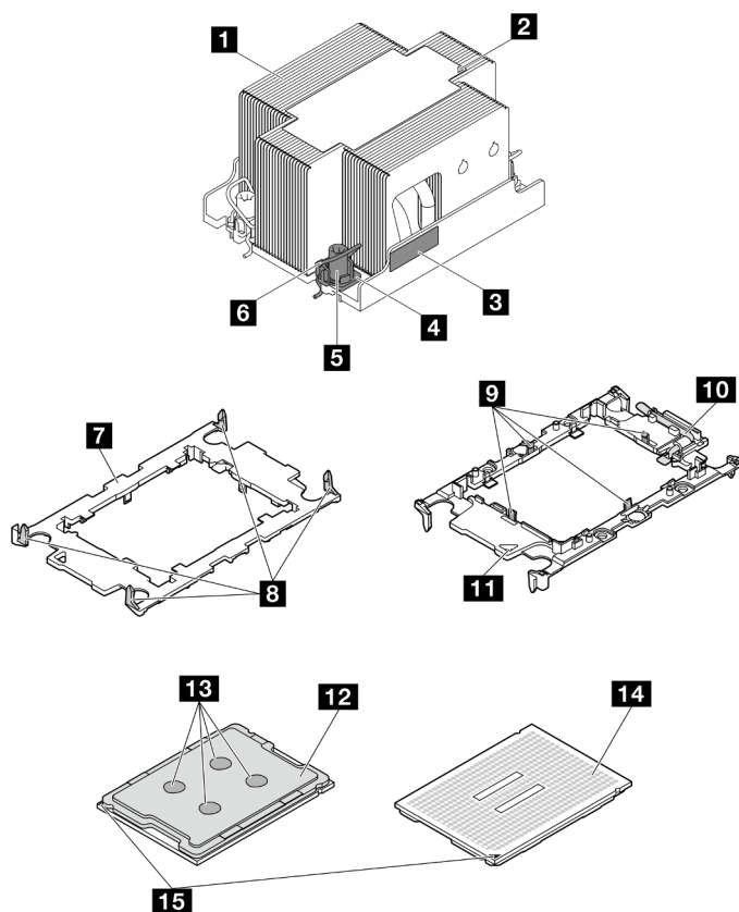
Figura 104. Componentes do PHM
