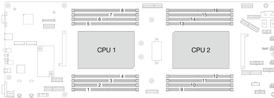
Figura 76. Layout de módulos de memória e processadores
