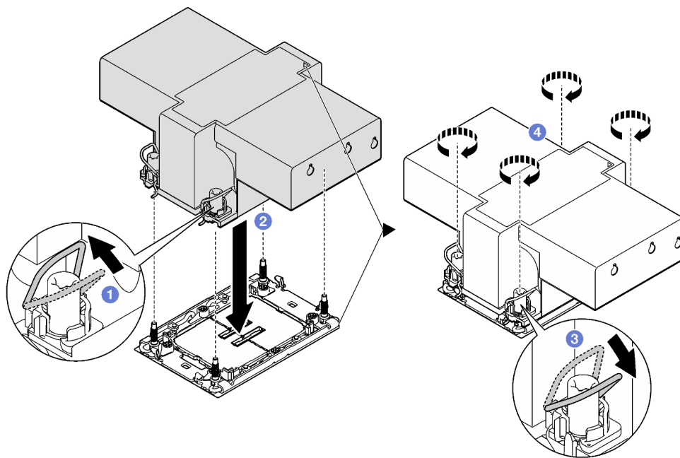
Figura 109. Instalação de um PHM de desempenho de 2U
