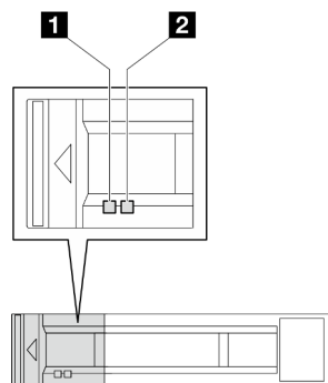
Figura 156. LEDs da unidade de 2,5"
