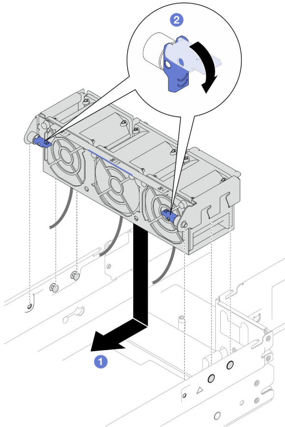
Figura 56. Instalação da gaiola do ventilador
