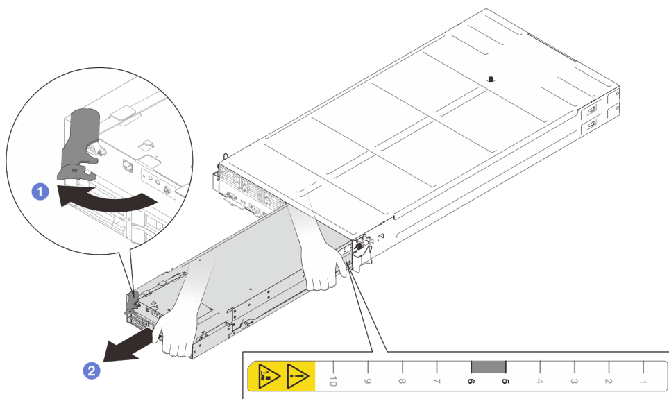
Figura 31. Remoção do nó da bandeja direita
