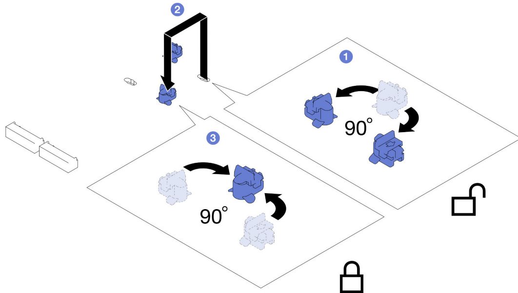
Figura 73. Ajuste de um retentor da unidade M.2
