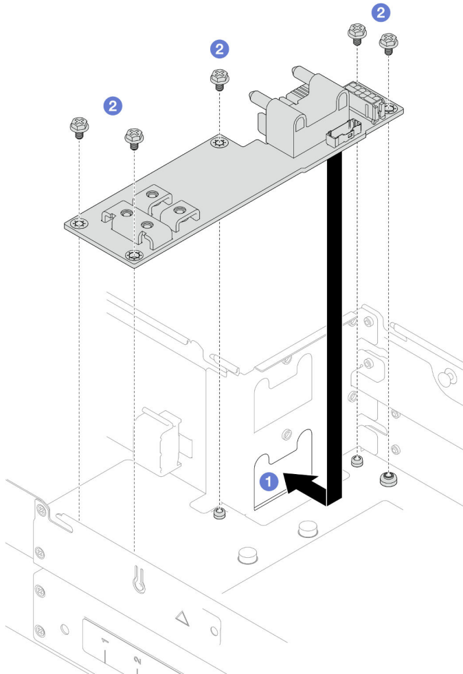
Figura 98. Instalação de uma placa de distribuição de energia
