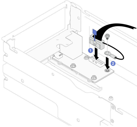
图 99. 安装背面 I/O 线缆和接地线缆
