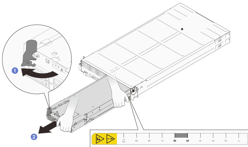
图 17. 将节点从右侧托盘卸下
