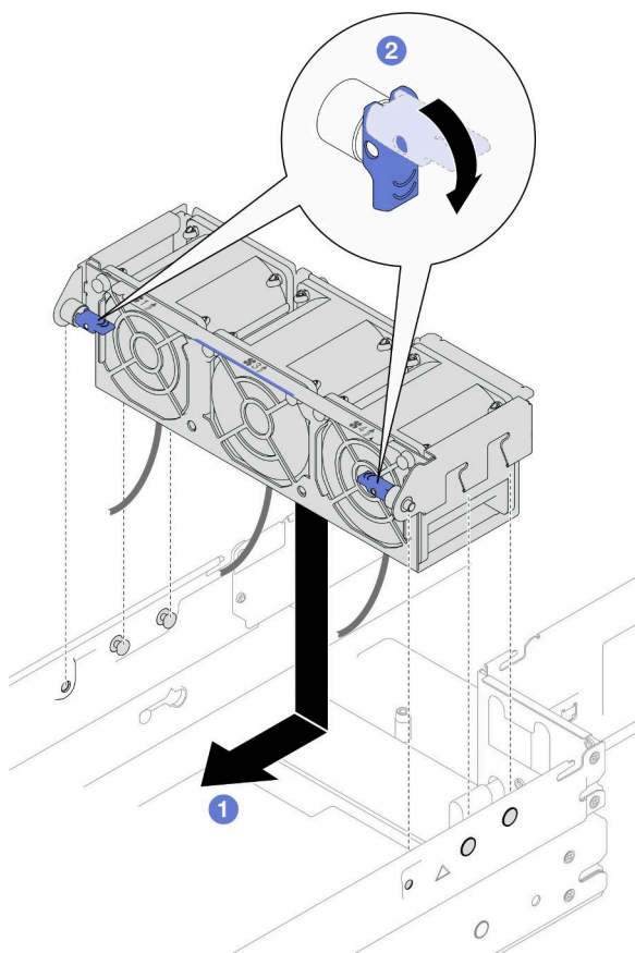
图 42. 安装风扇架
