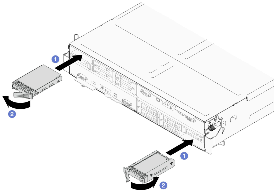
图 53. 安装 7 毫米固态硬盘
