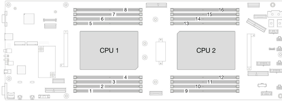
图 62. 内存条和处理器布局
