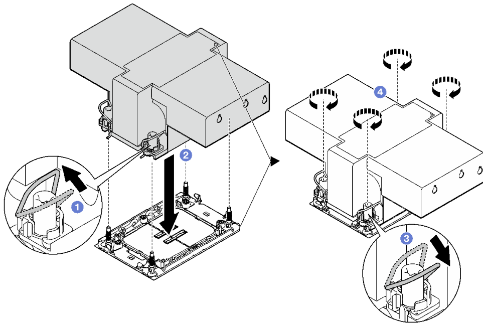
图 95. 安装 2U 高性能 PHM
