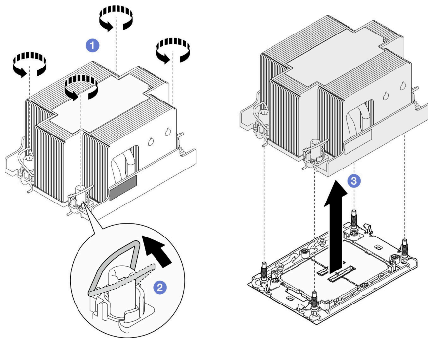
图 86. 卸下 2U 标准 PHM
