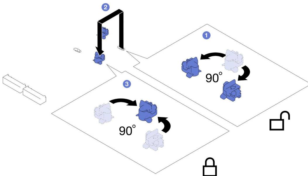
图 59. 调整 M.2 硬盘固定器
