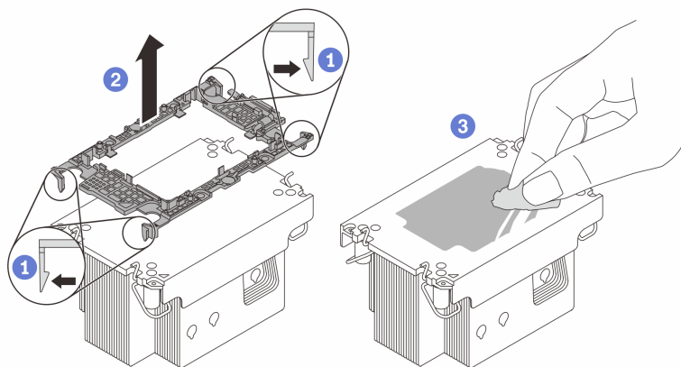
图 89. 将处理器支架与散热器分开
