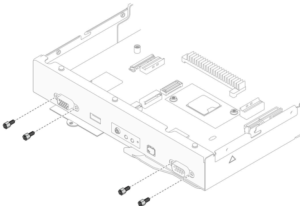
图 111. 安装正面的主板螺钉
