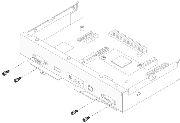
图 107. 卸下螺钉
