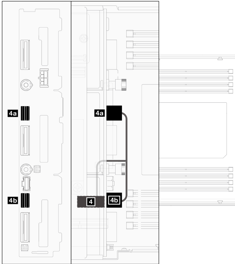
图 123. SATA 线缆布放 – 不带 CFF RAID 的配置
