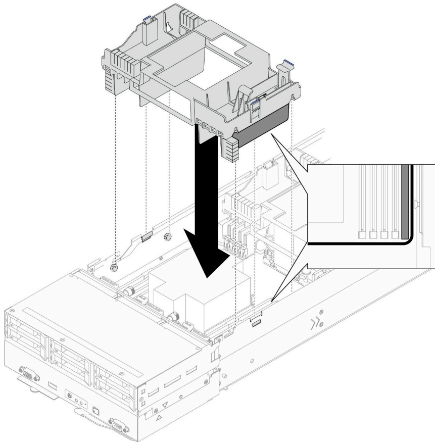
图 26. 安装正面导风罩
