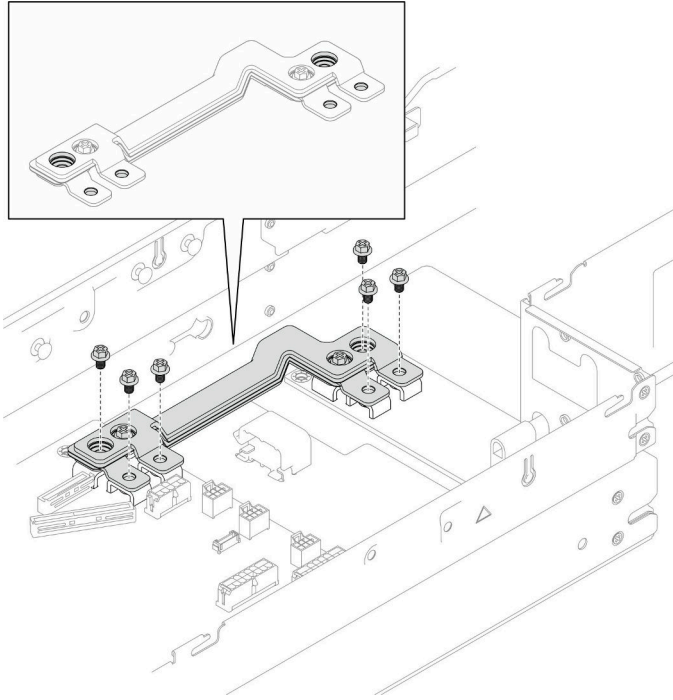
图 79. 卸下电源汇流条外侧螺钉
