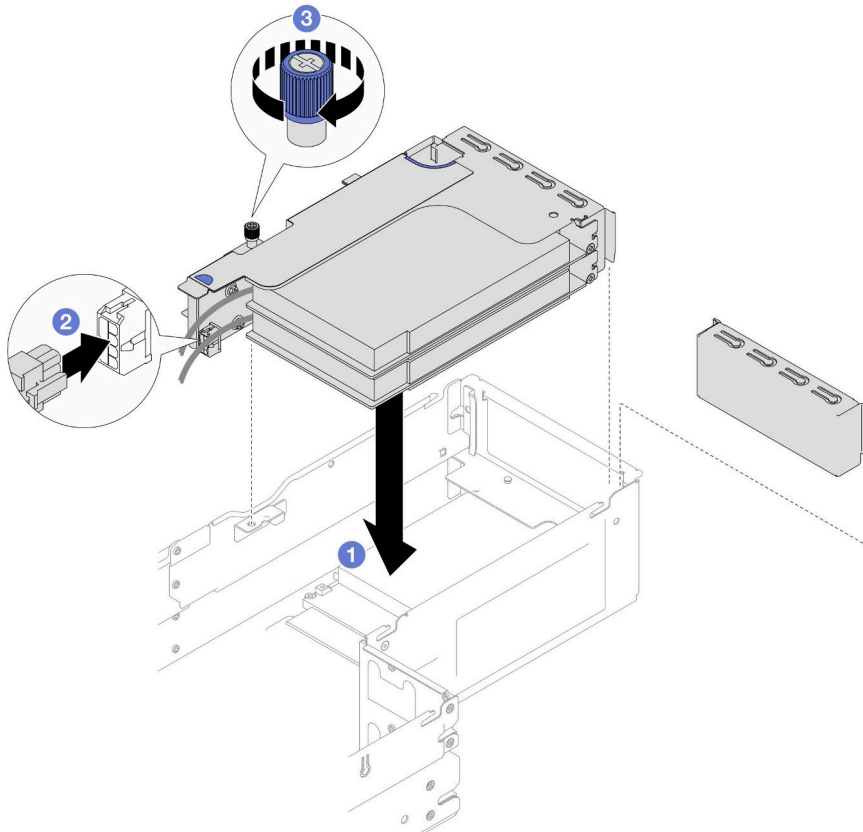
图 78. 安装 PCIe 转接卡组合件
