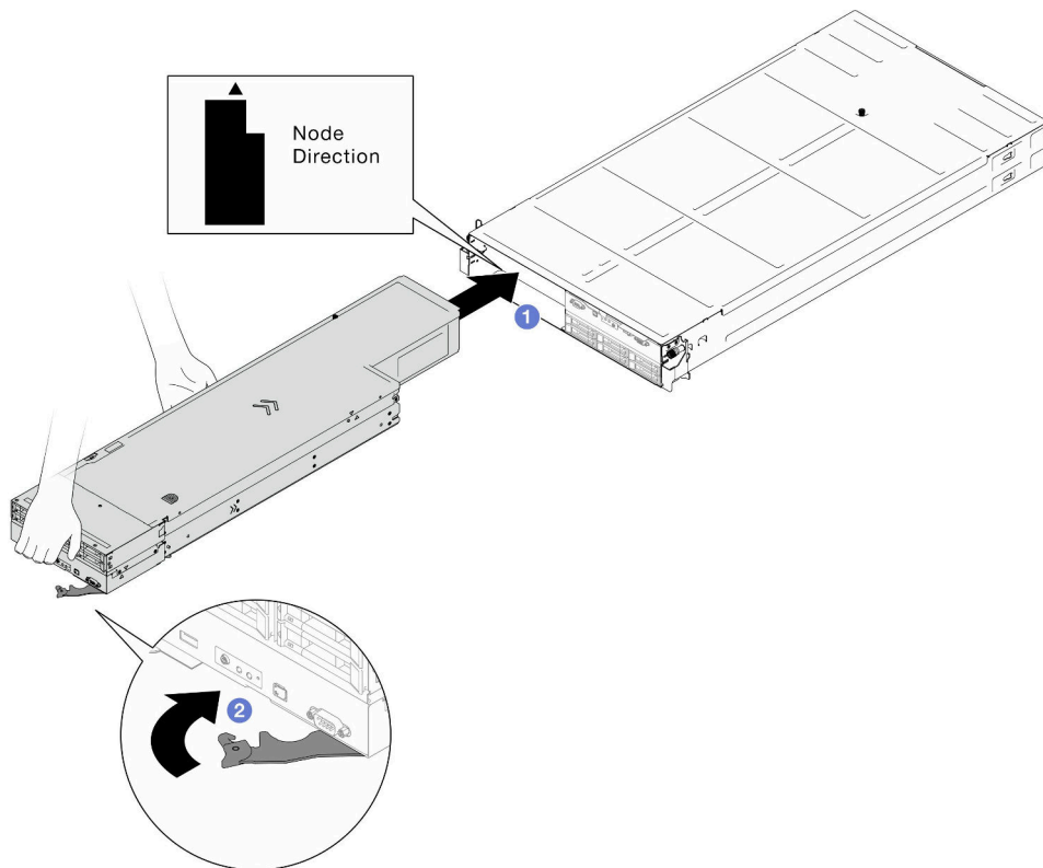
图 22. 将节点安装到左侧托盘
