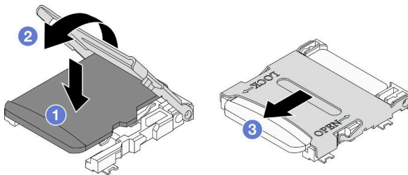
图 69. 安装 MicroSD 卡
