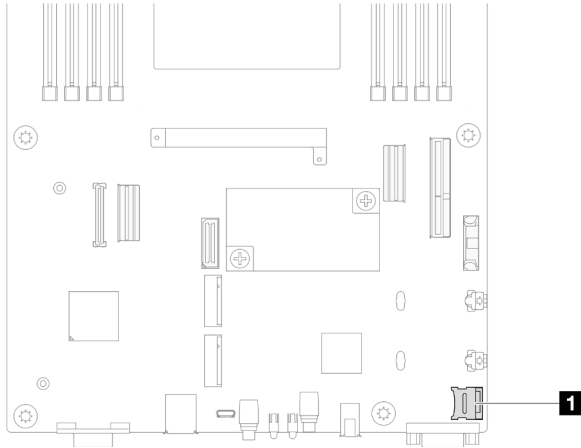
图 68. MicroSD 插槽位置
