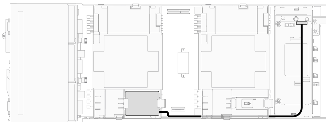
图 129. CFF RAID 和快速充电模块线缆
