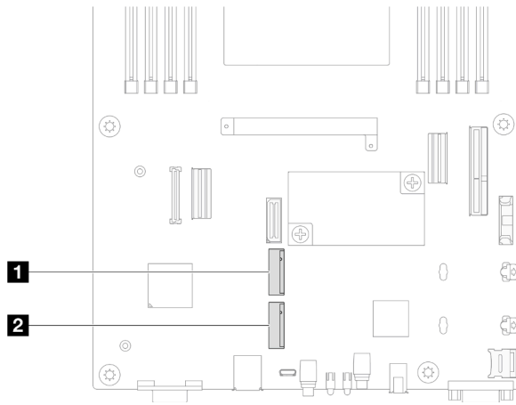
图 57. 主板上 M.2 插槽的位置
