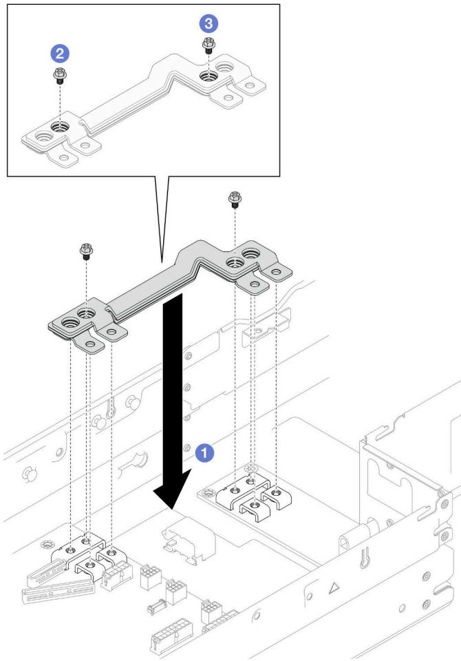
图 81. 安装电源汇流条
