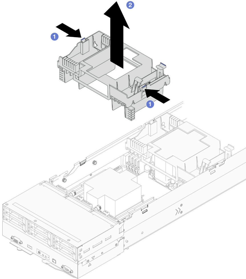
图 24. 卸下正面导风罩
