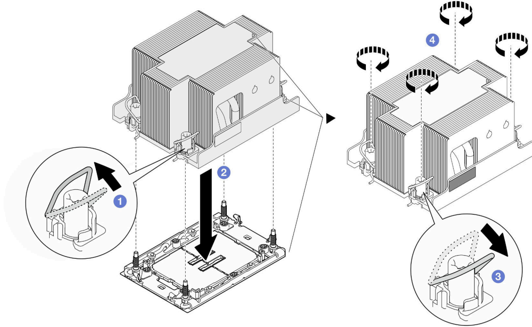
图 94. 安装 2U 标准 PHM
