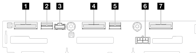
图 116. 2.5 英寸硬盘背板
