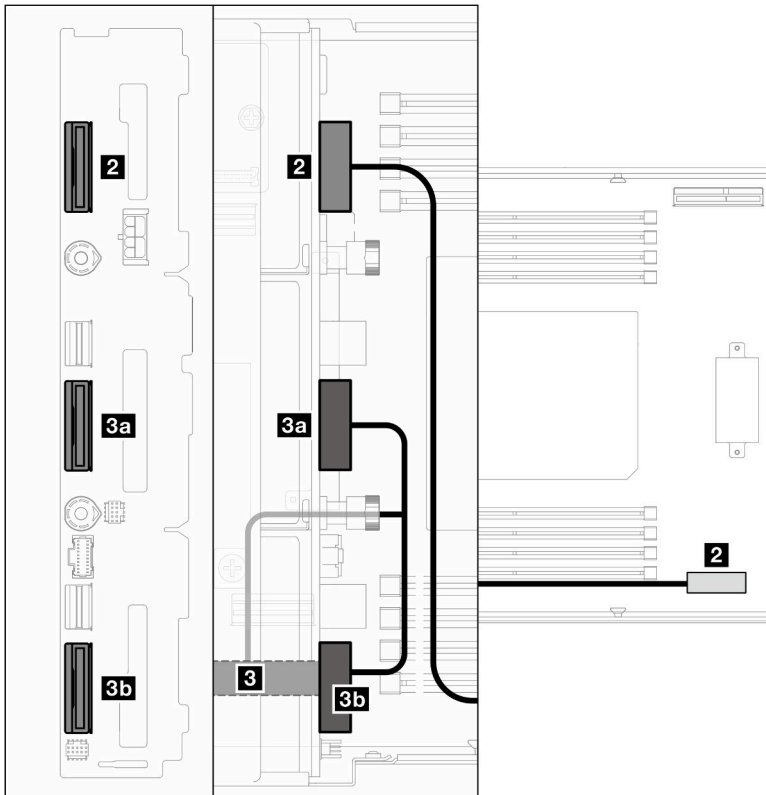
图 125. NVMe 线缆布放
