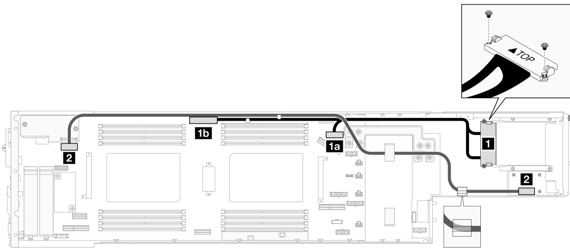
图 133. 背面 I/O 模块和 OCP 模块的线缆
