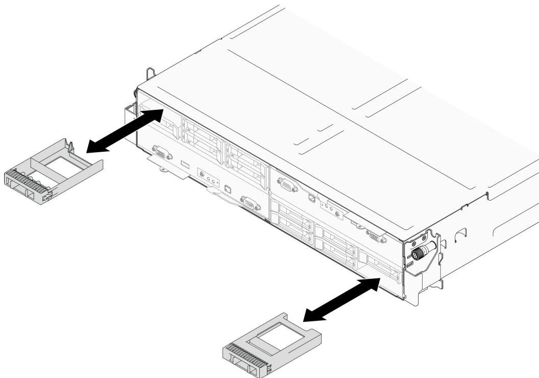
图 52. 更换硬盘填充件
