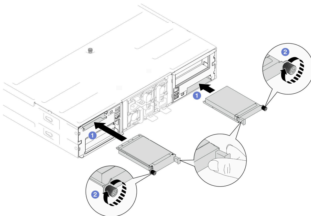
图 71. 安装背面 OCP 模块
