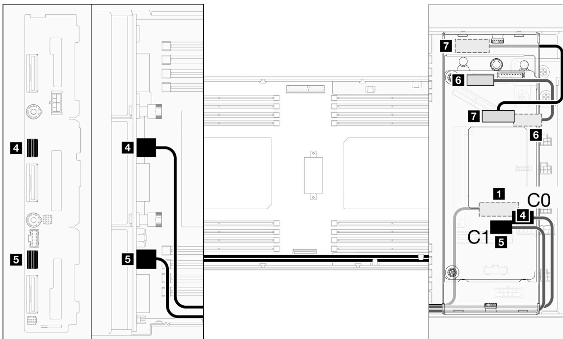
图 127. SATA 和 CFF RAID 线缆布放
