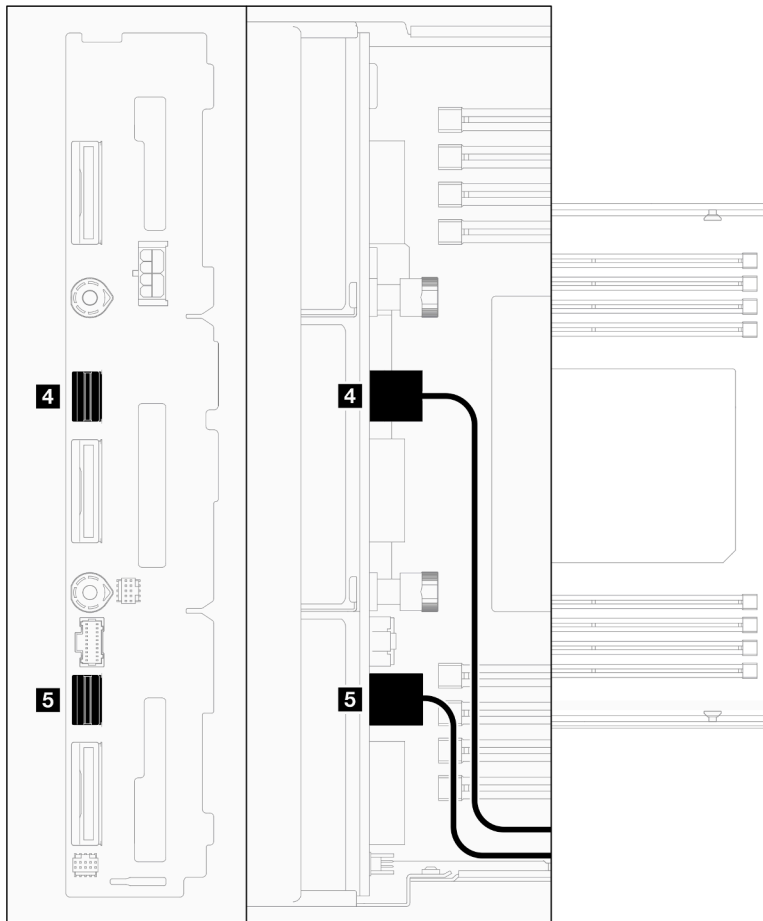
图 126. 硬盘背板上的 SATA 线缆
