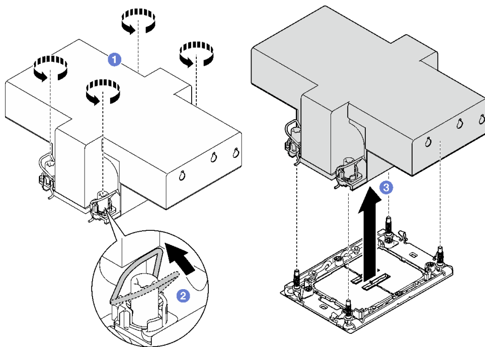
图 87. 卸下 2U 高性能 PHM
