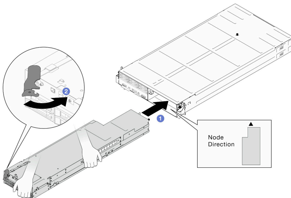
图 23. 将节点安装到右侧托盘
