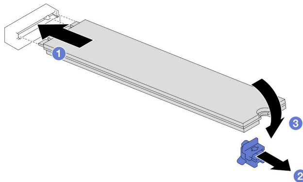
图 61. 安装 M.2 硬盘
