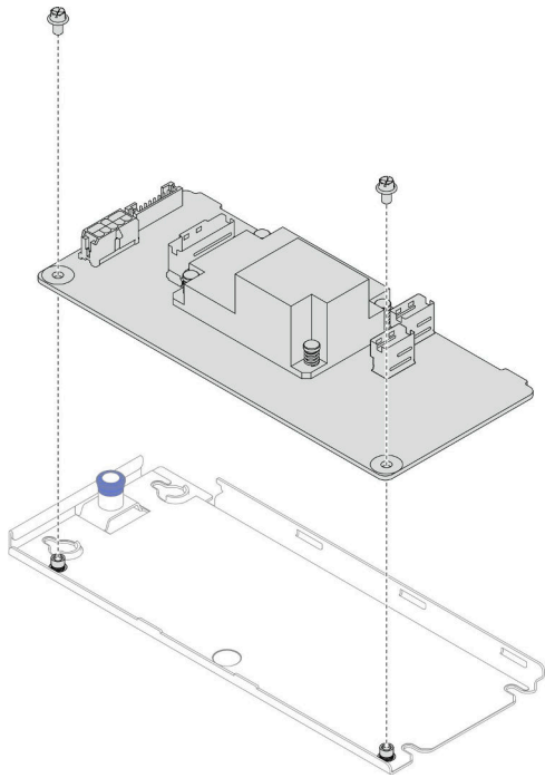
图 29. 将内部 CFF RAID 适配器与托盘分开
