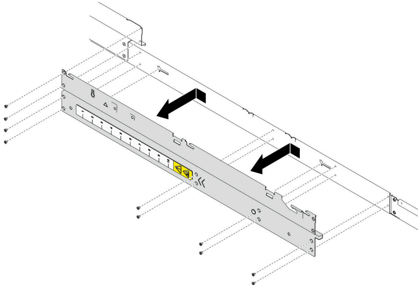
图 100. 卸下侧支架
