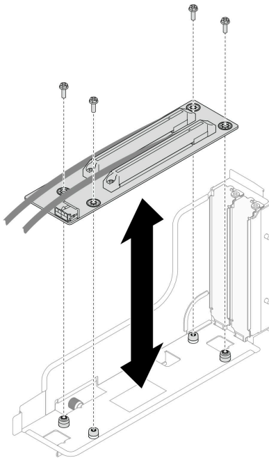
图 73. 更换 PCIe 转接卡
