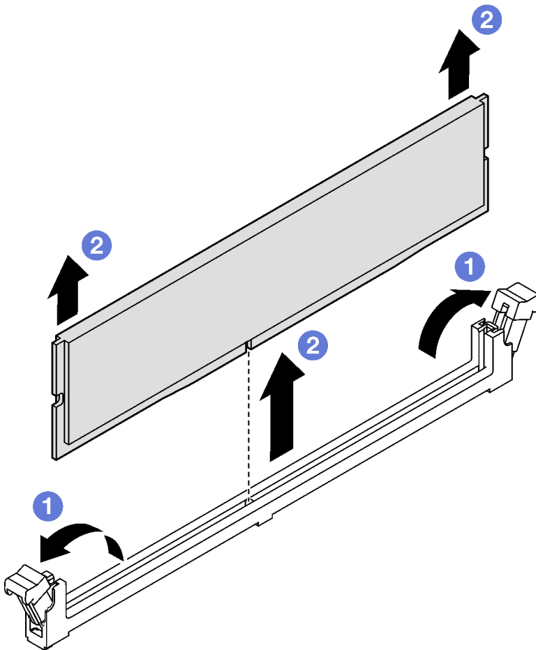
图 63. 卸下内存条
