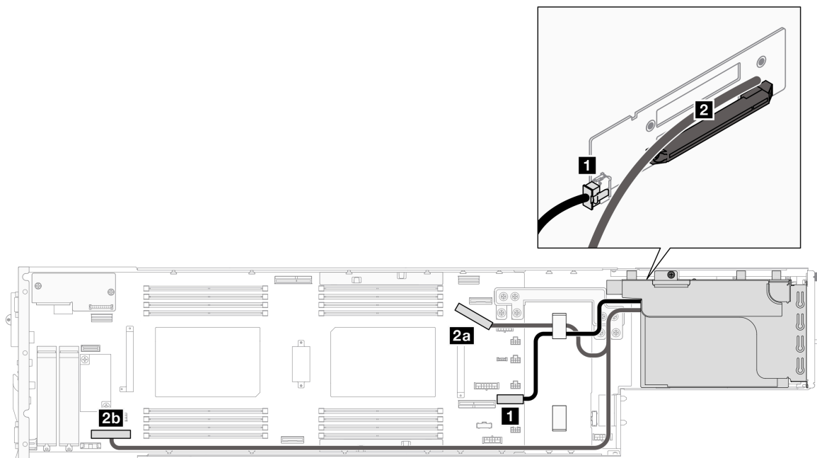
图 130. PCIe 转接卡线缆布放 - 一个处理器
