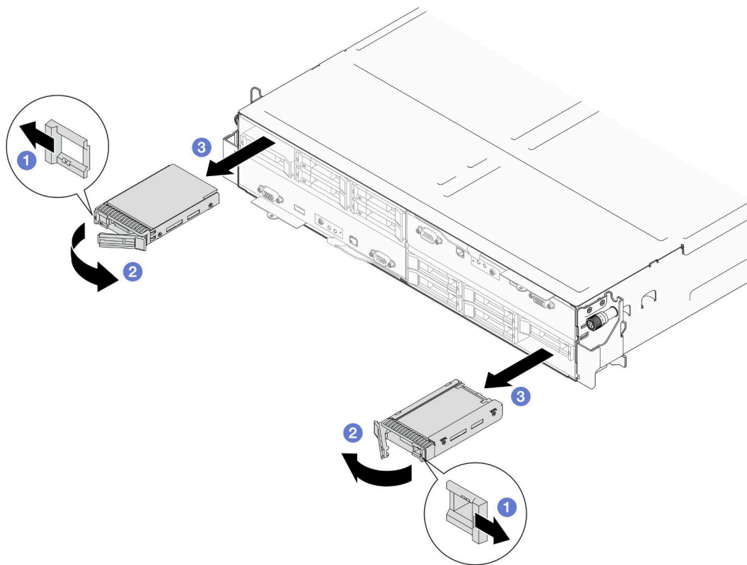
图 50. 卸下 15 毫米固态硬盘
