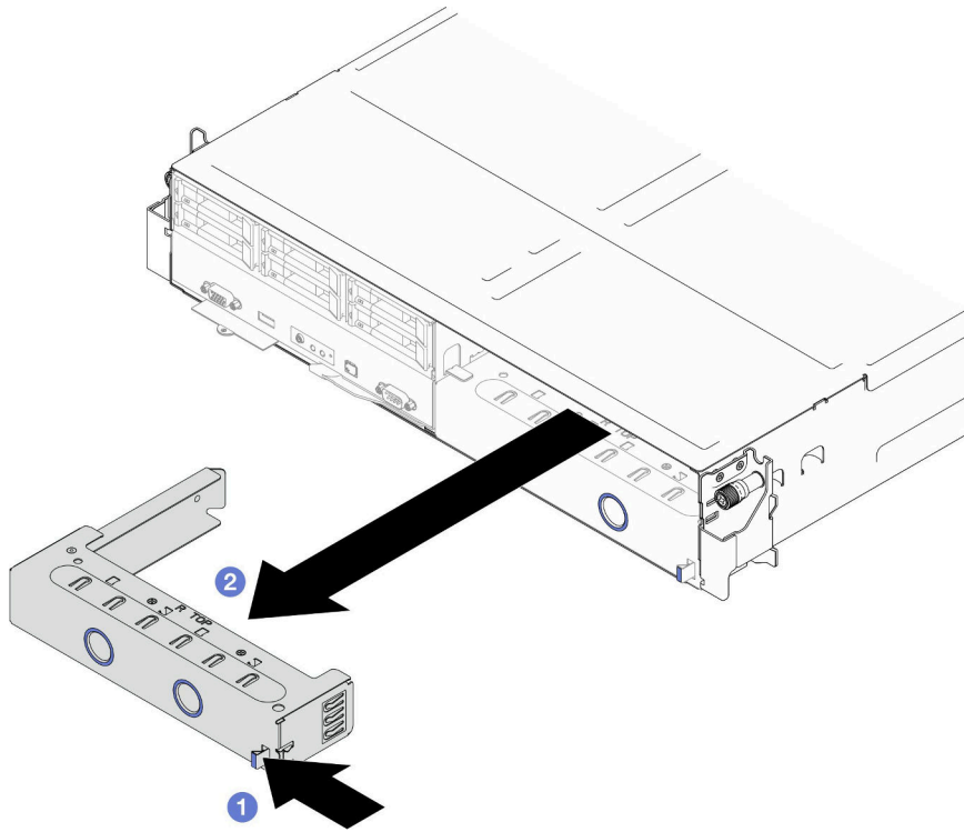
图 20. 卸下正面节点托盘填充件
