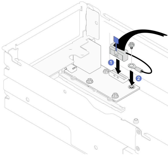
图 134. 安装背面 I/O 线缆和接地线缆
