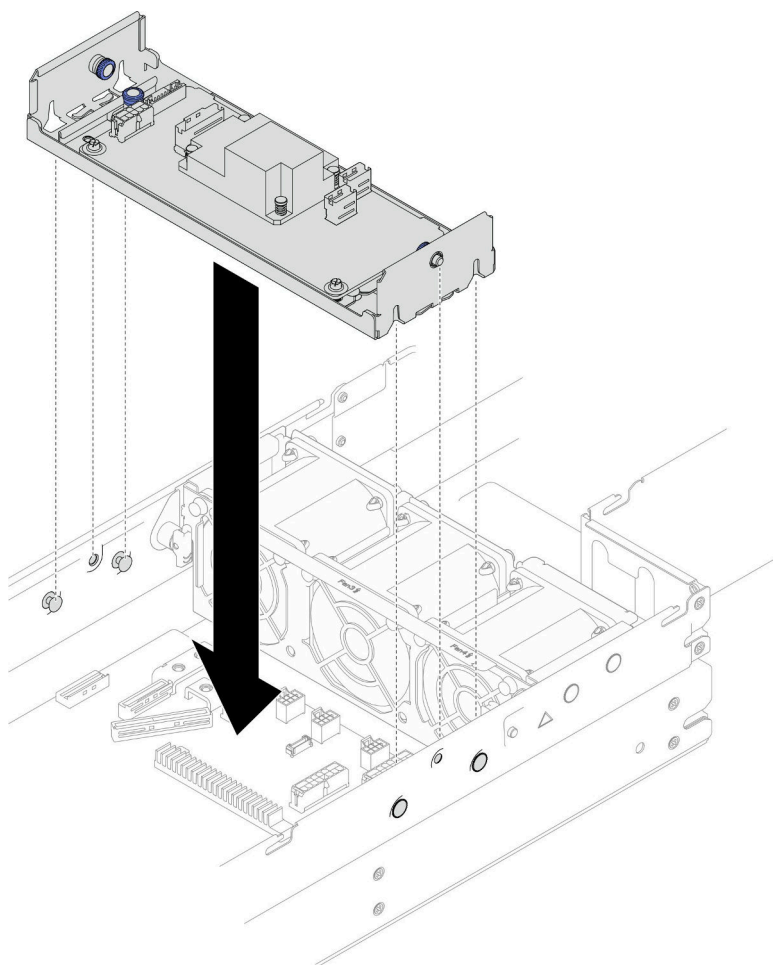
图 56. 安装内部适配器支架
