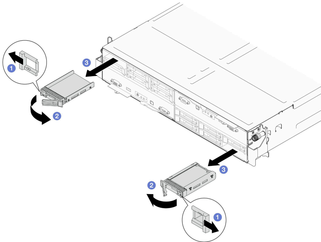
图 49. 卸下 7 毫米固态硬盘
