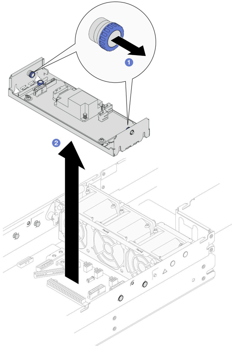
图 55. 卸下内部适配器支架
