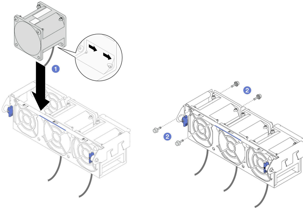
图 41. 安装风扇
