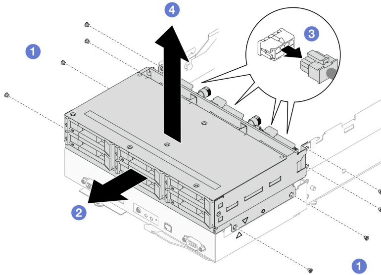
图 35. 卸下硬盘仓组合件
