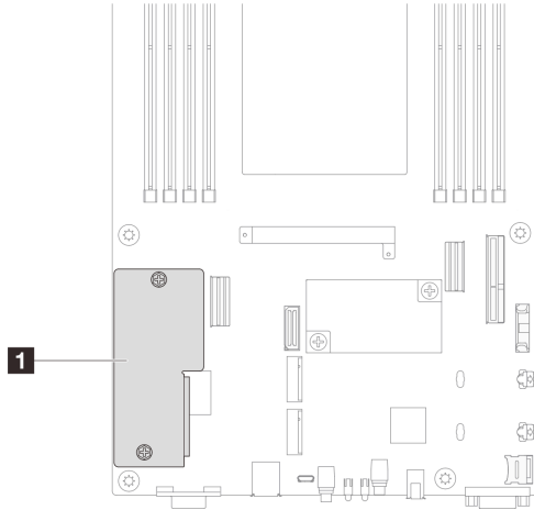
图 102. 固件和 RoT 安全模块位置
