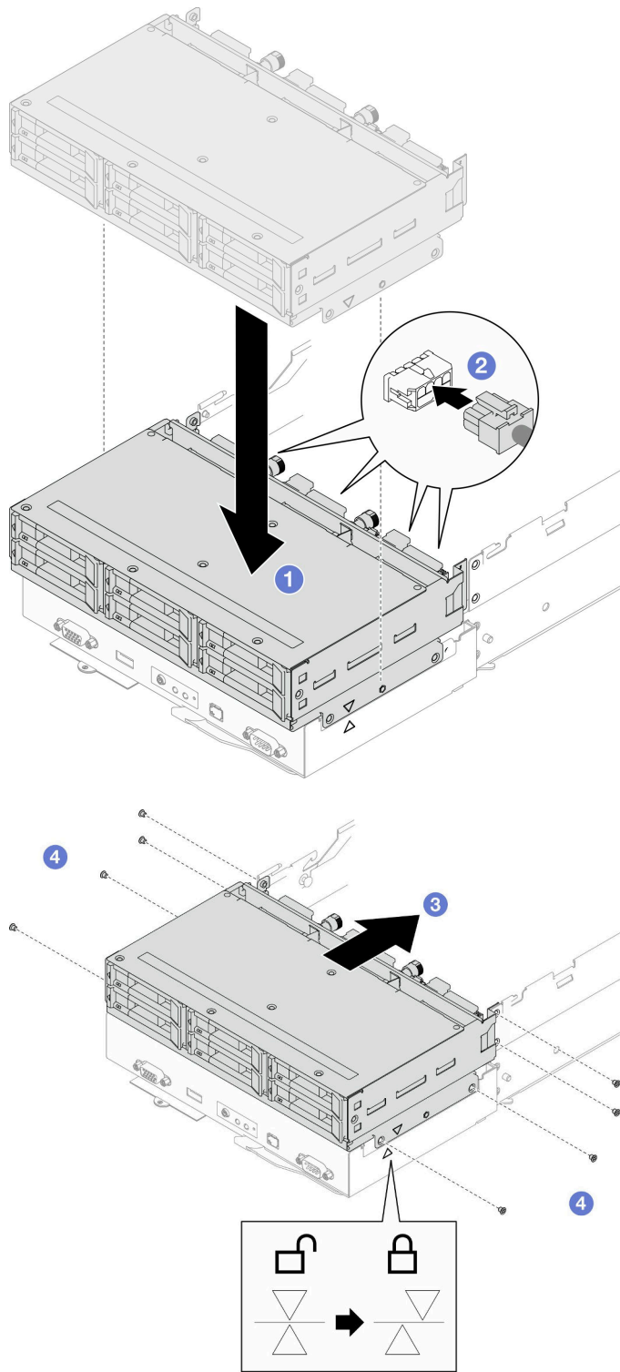
图 38. 安装硬盘仓组合件
