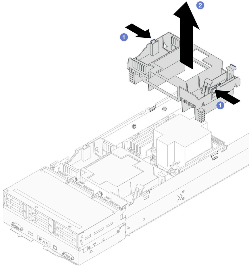
图 25. 卸下背面导风罩
