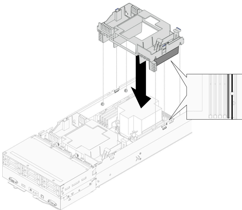
图 27. 安装背面导风罩
