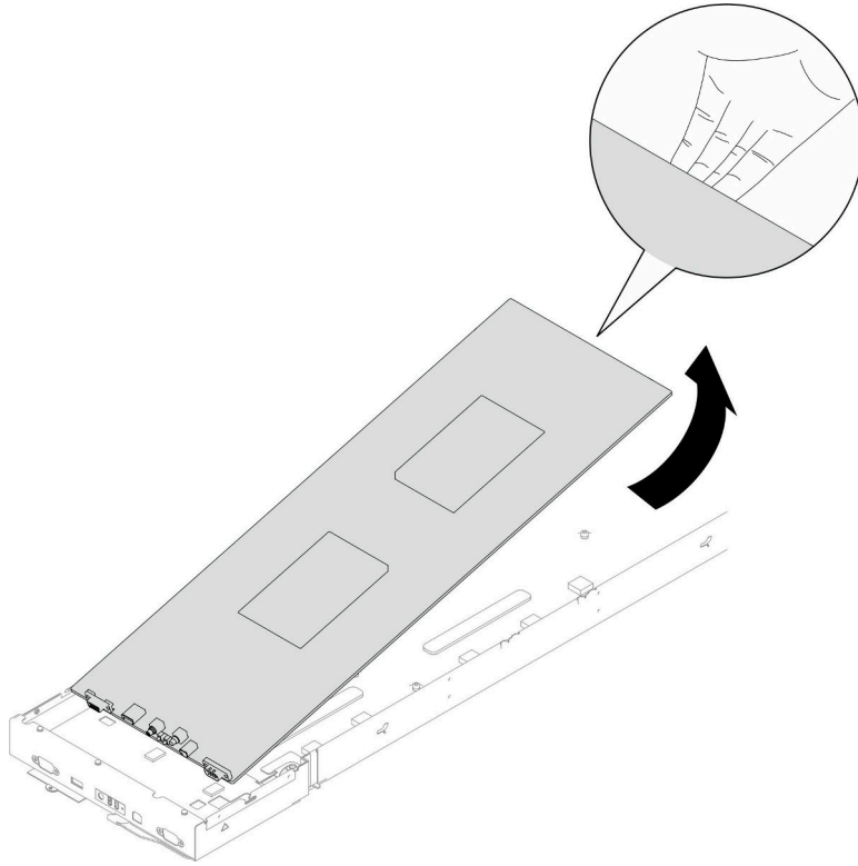
图 109. 卸下主板
