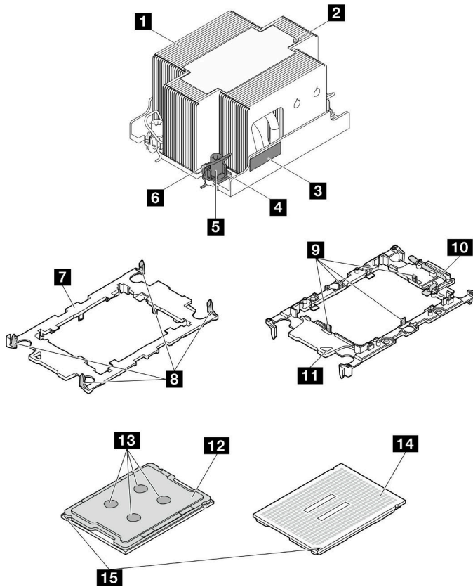
图 85. PHM 组件
