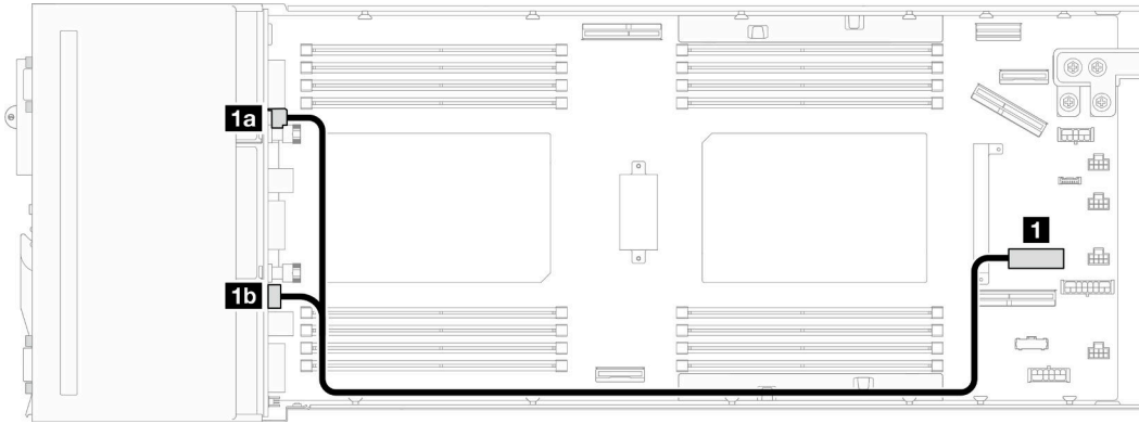
图 124. 硬盘背板电源线布放
