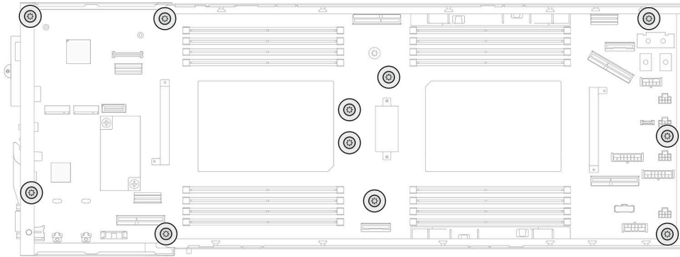
图 108. 卸下螺钉
