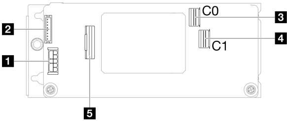
图 117. 内部 CFF RAID 适配器接口
