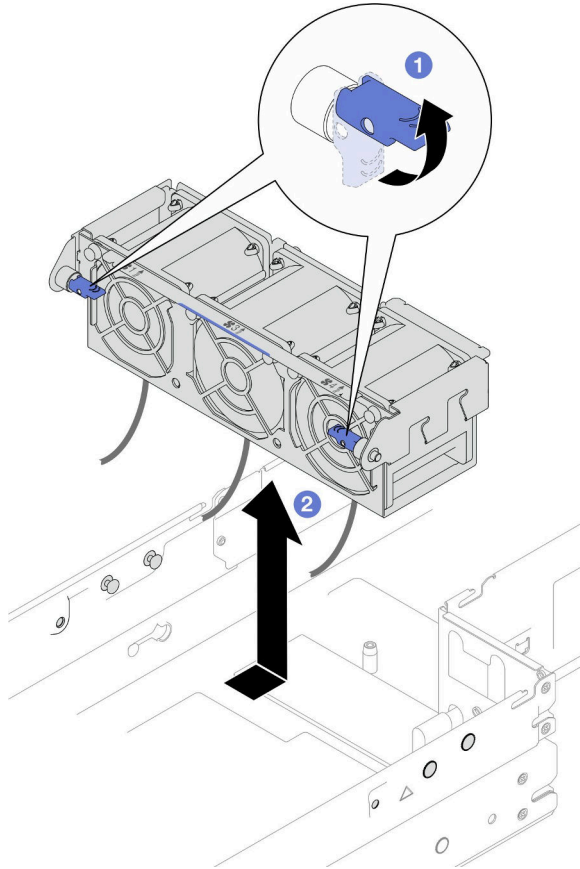
图 39. 卸下风扇架
