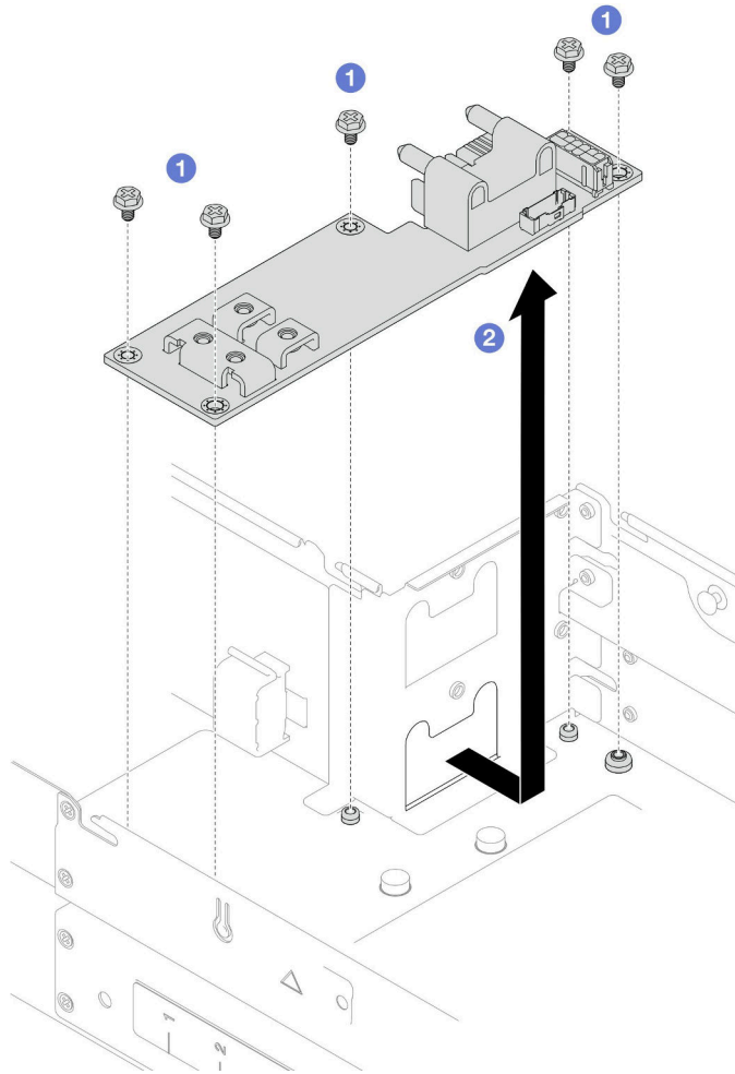
图 83. 卸下配电板
