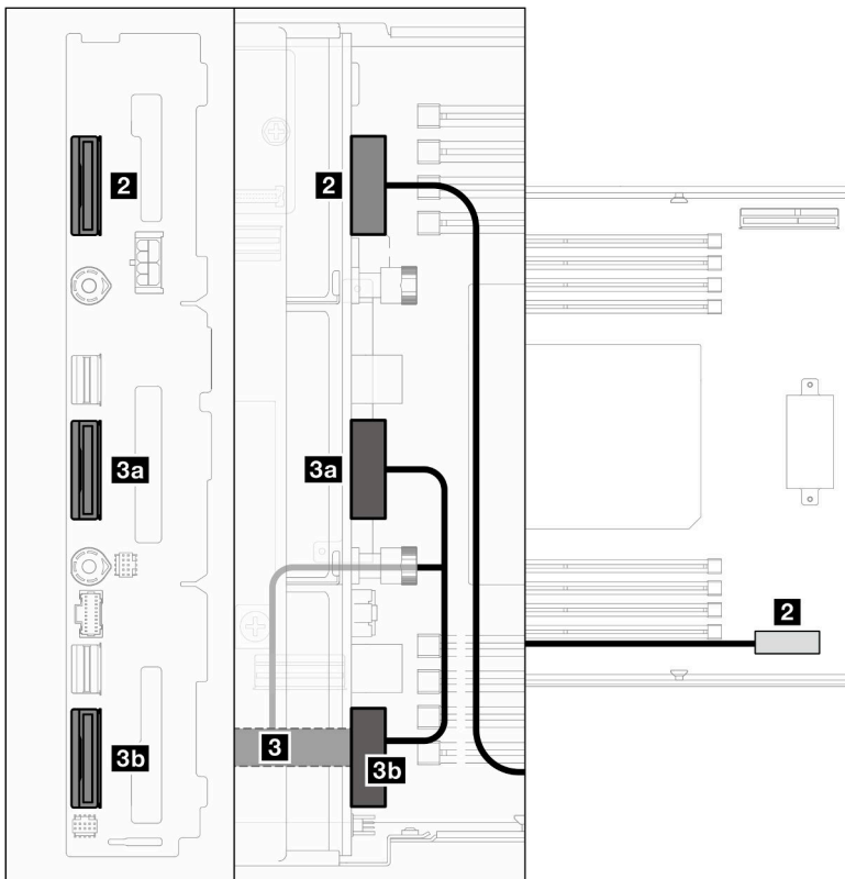
图 122. NVMe 线缆布放
