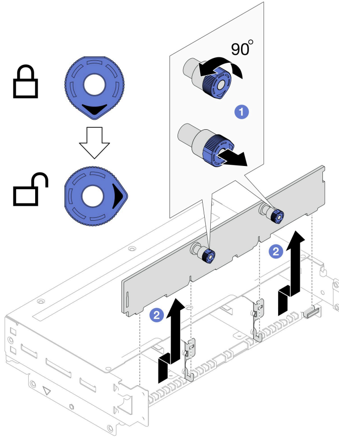
图 36. 卸下硬盘背板
