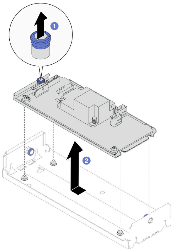
图 28. 卸下内部 CFF 适配器
