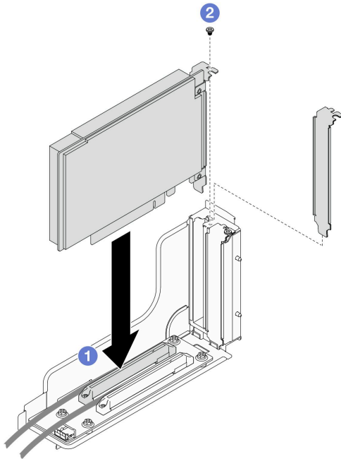
图 76. 安装 PCIe 适配器
