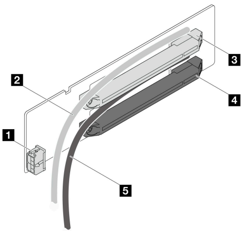
图 119. 双插槽 PCIe 转接卡接口和线缆
