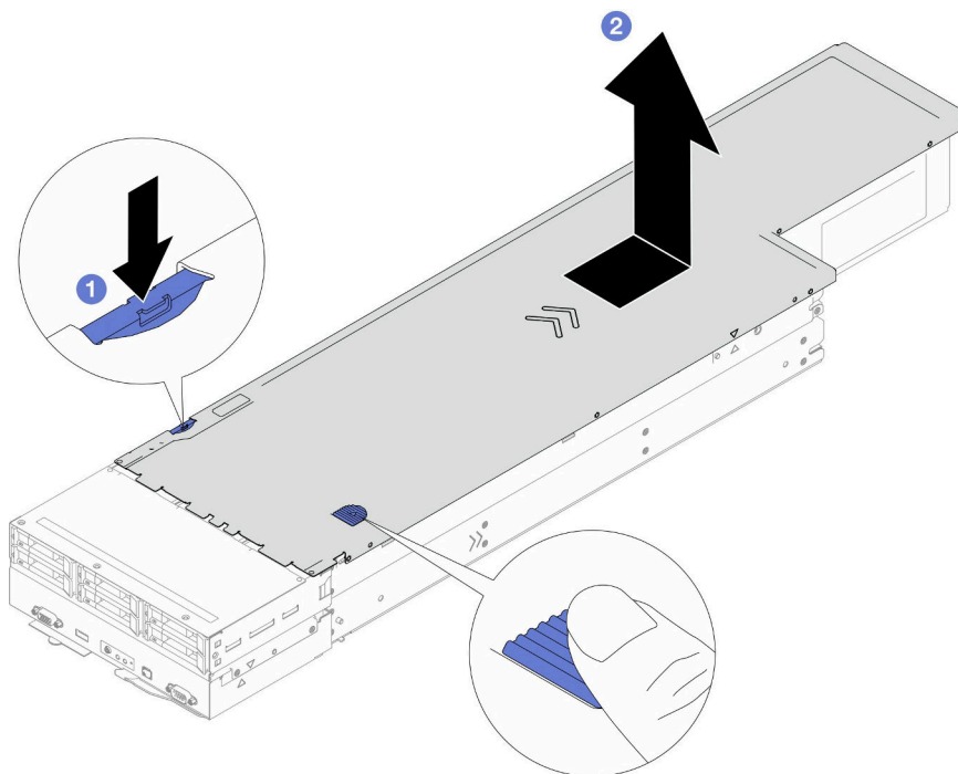
图 114. 卸下顶盖
