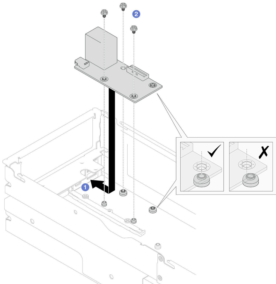
图 98. 安装背面 I/O 模块
