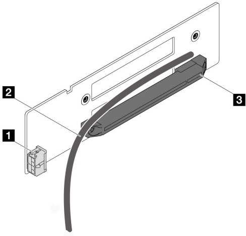
图 118. 单插槽 PCIe 转接卡接口和线缆
