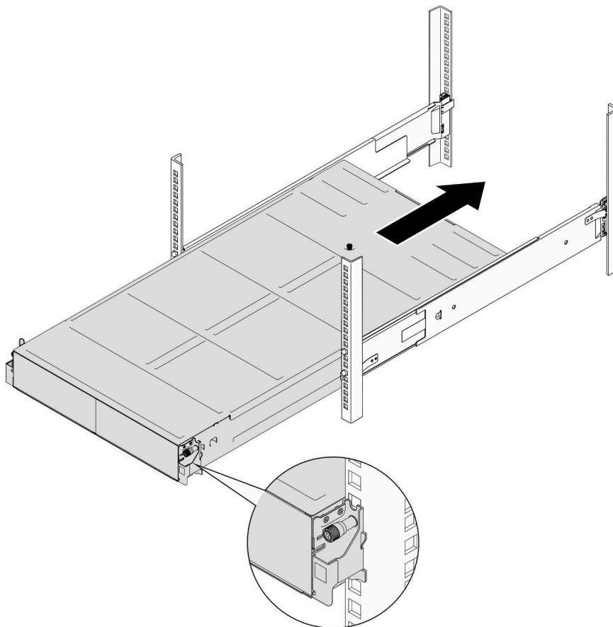
图 4. 安装机箱
