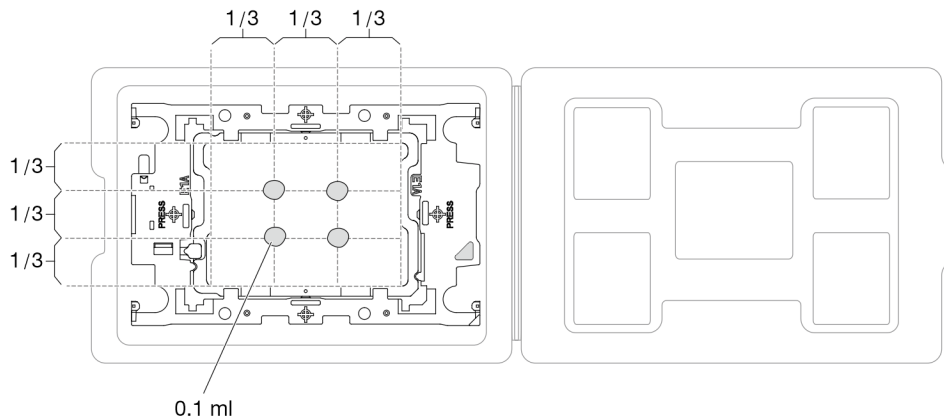
图 92. 为装运托盘中的处理器涂抹导热油脂
