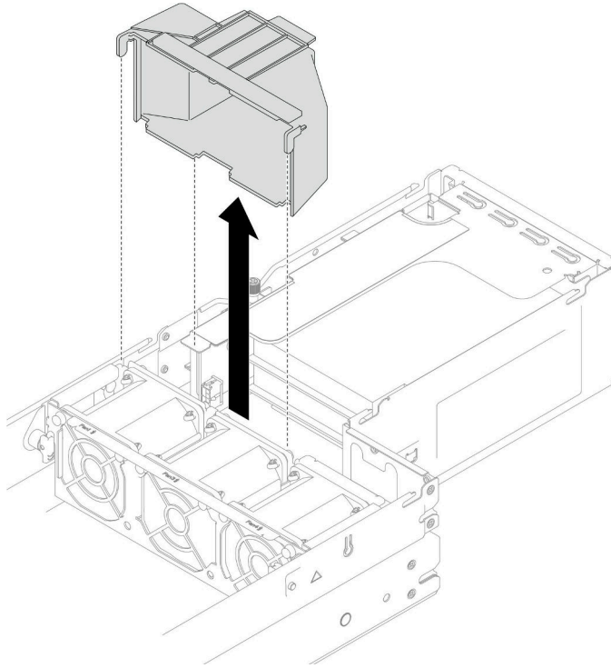
图 47. 卸下 GPU 导风管
