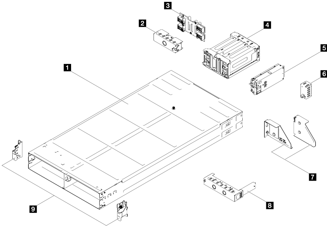
图 15. 机箱组件
