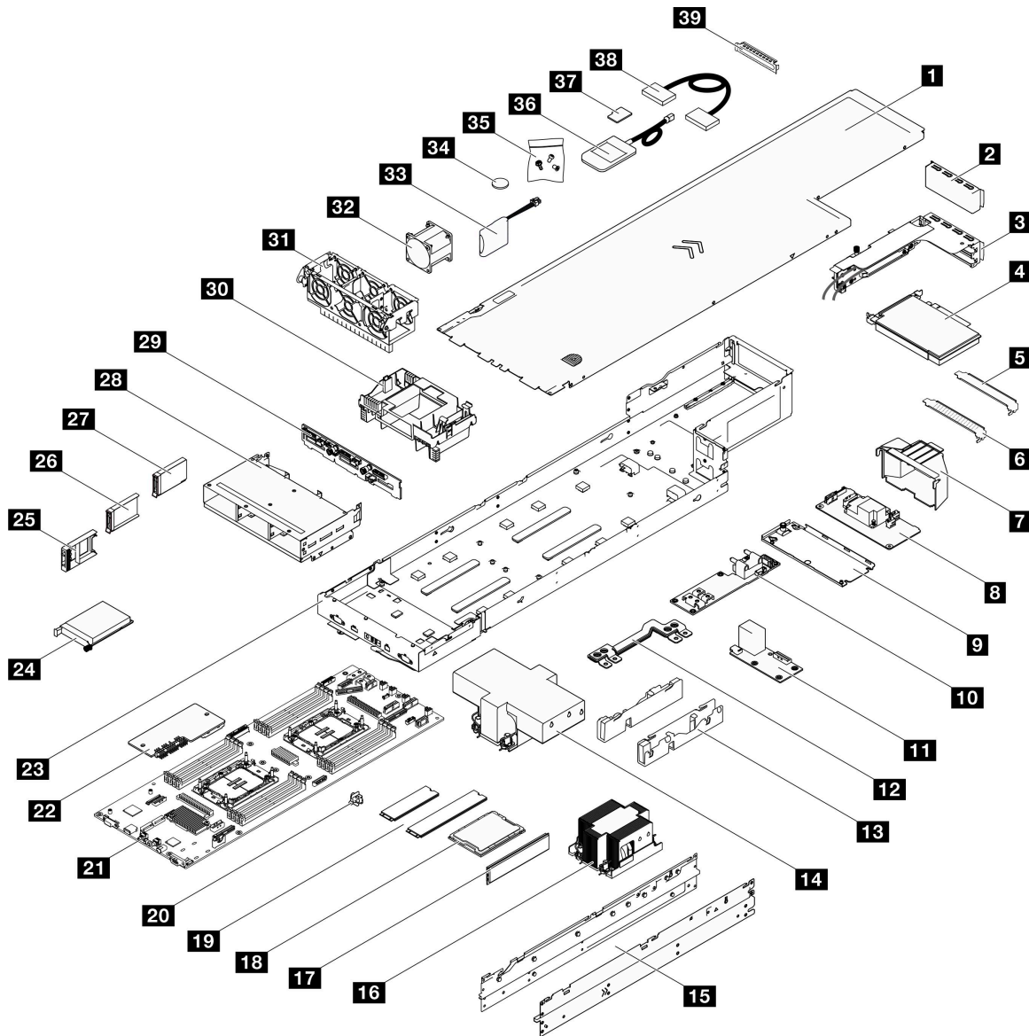
图 16. 节点组件
