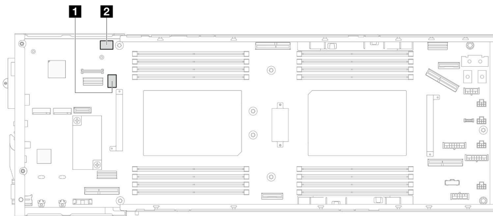
图 9. 主板开关
