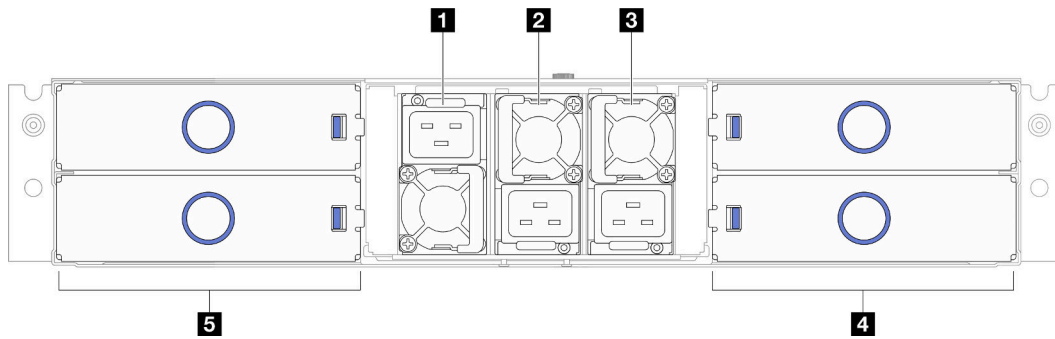
图 3. 机箱后视图
