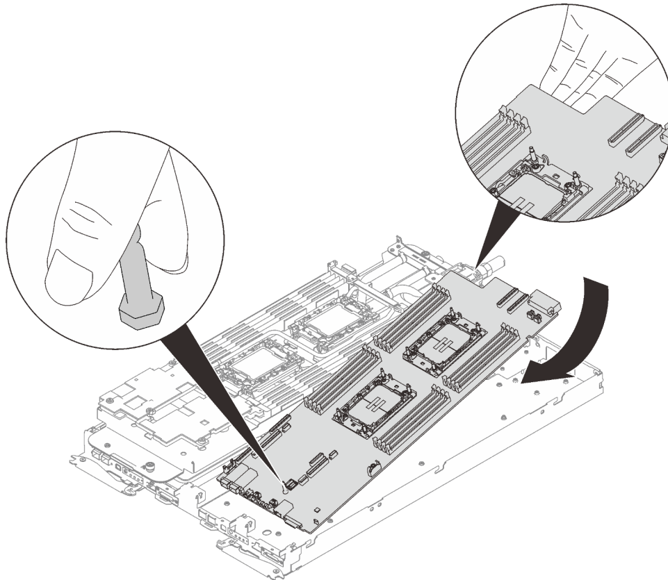
Figure 251. Installation de la carte mère
