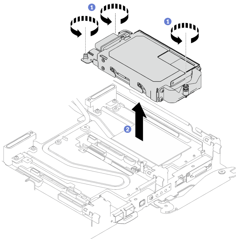
Figure 115. Retrait du bloc boîtier d'unités de disque dur E3.S
