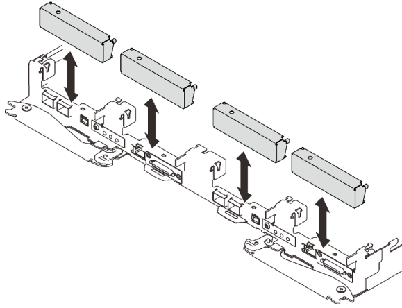
Figure 185. Retrait de l'obturateur vide du panneau
