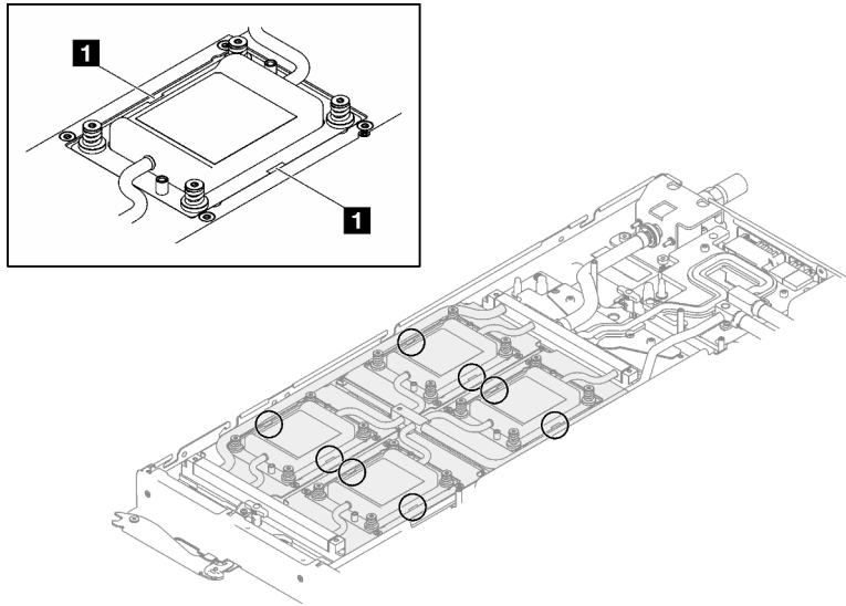
Figure 259. Encoches sur la plaque froide du GPU OAM
