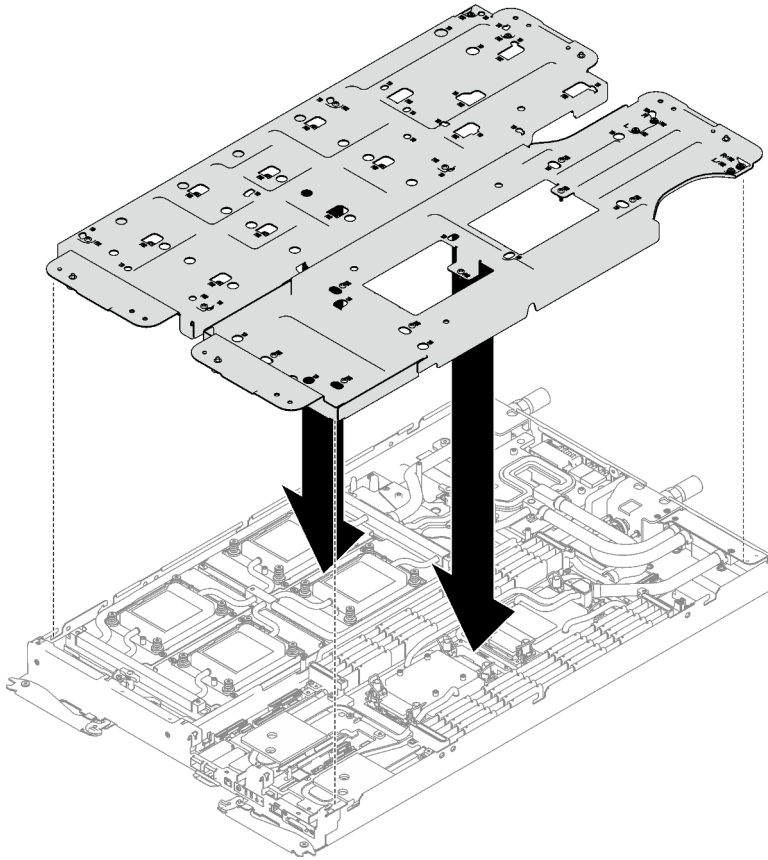
Figure 33. Installation du support de boucle d'eau
