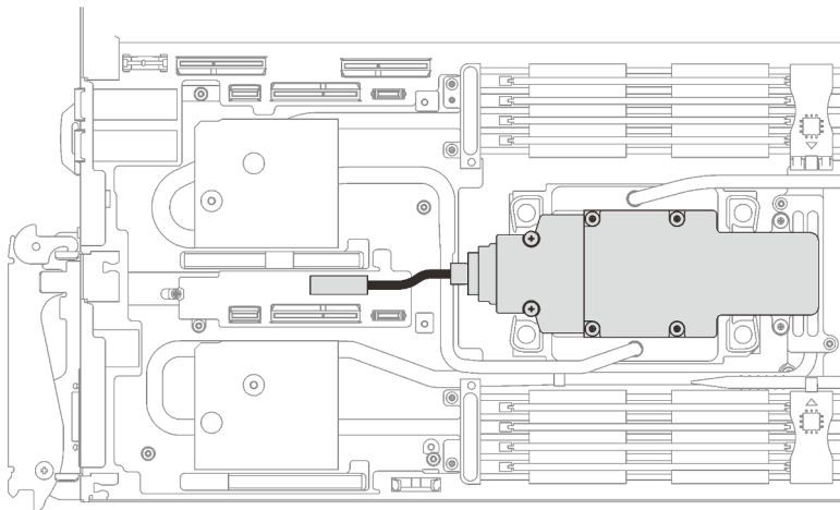
Figure 148. Installation du câble du fond de panier M.2
