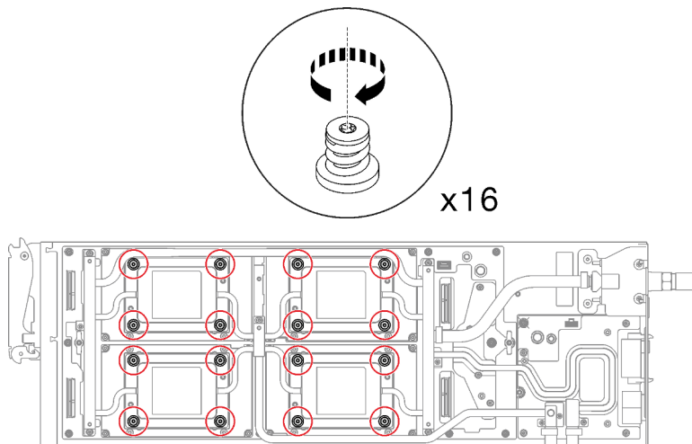
Figure 317. Installation des vis de la plaque froide du GPU OAM
