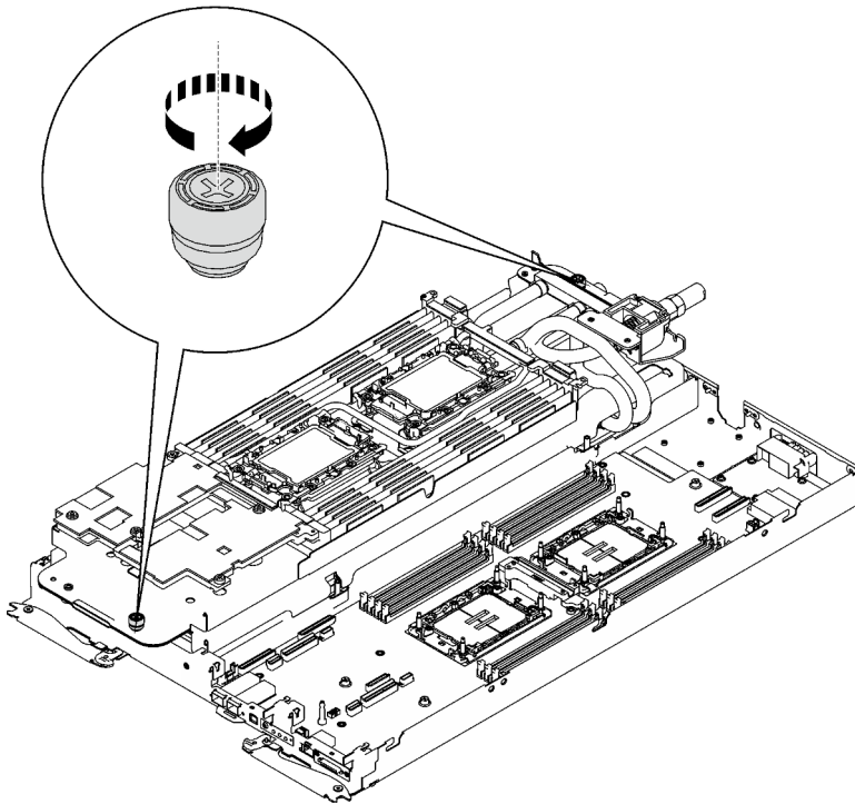
Figure 36. Serrage des vis moletées imperdables
