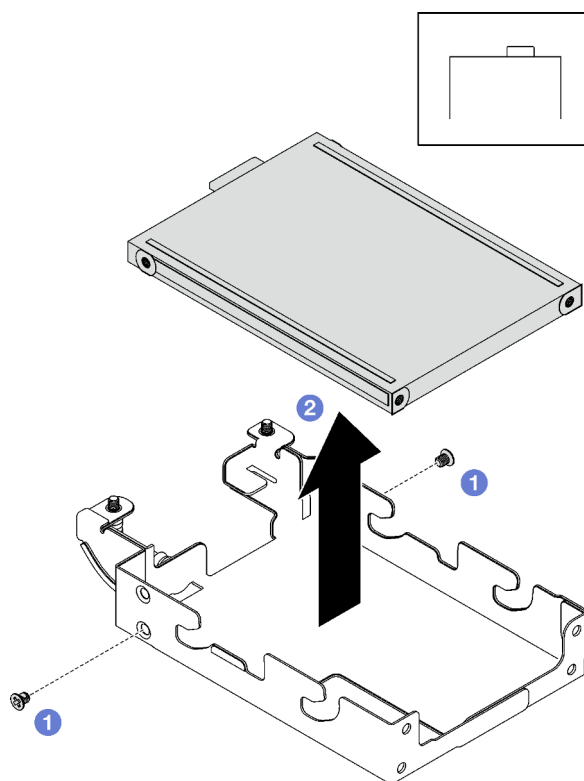
Figure 122. Retrait de l'unité E3.S supérieure
