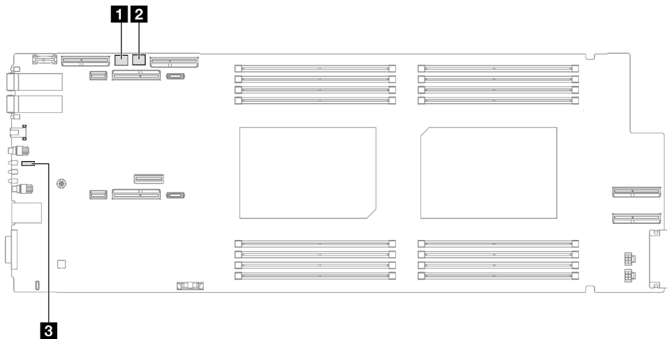
Figure 8. Commutateurs sur la carte mère du nœud de traitement
