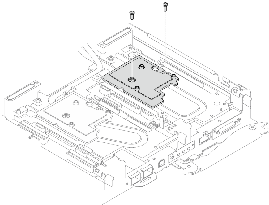
Figure 193. Retrait de la plaque d'interface
