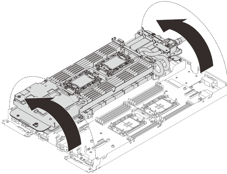
Figure 227. Plier la boucle d'eau
