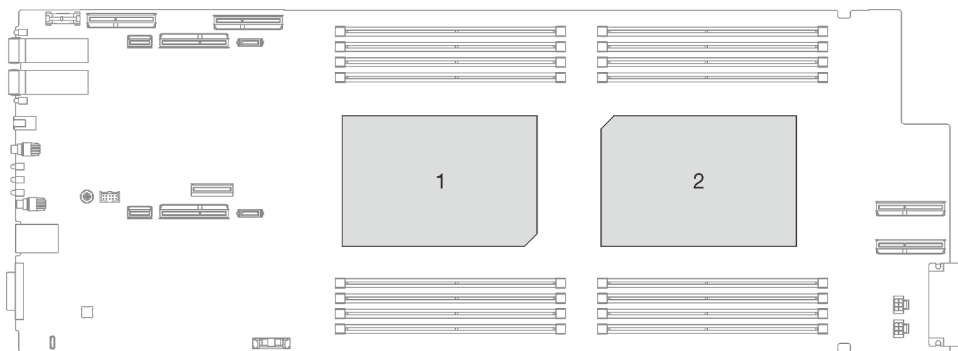
Figure 220. Emplacements des processeurs
