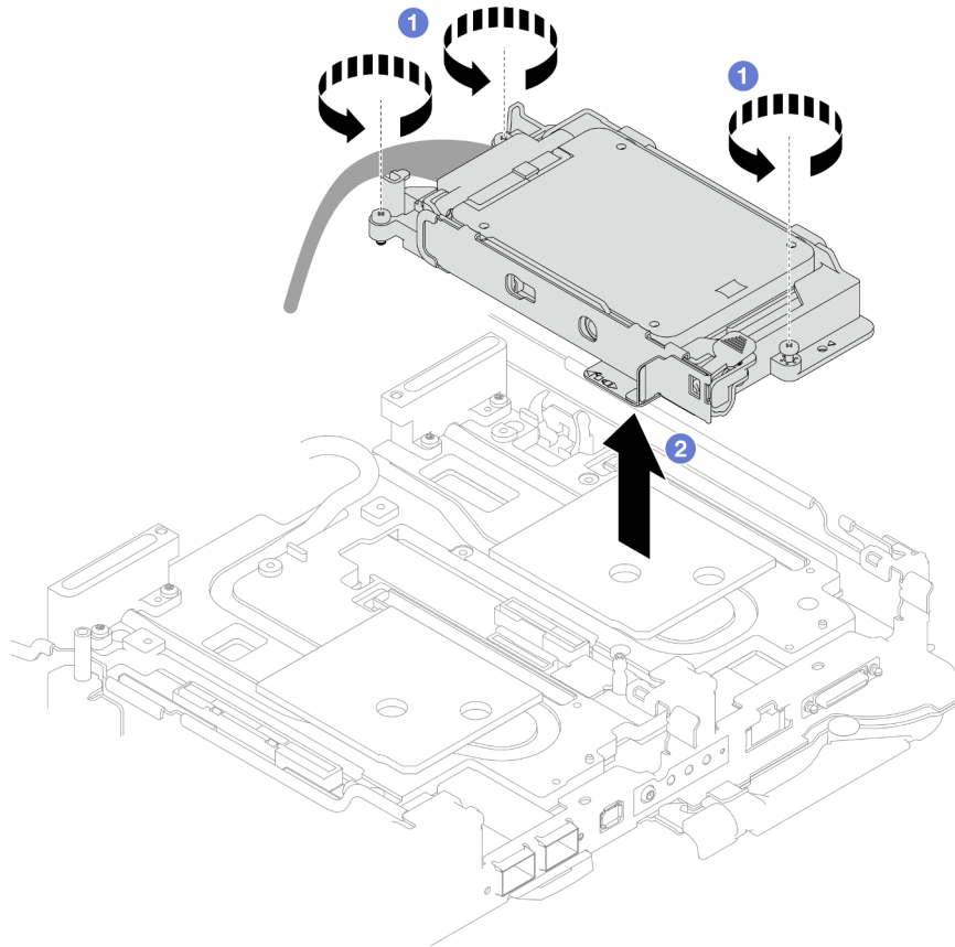
Figure 100. Retrait du bloc boîtier d'unités de disque dur NVMe 7 mm
