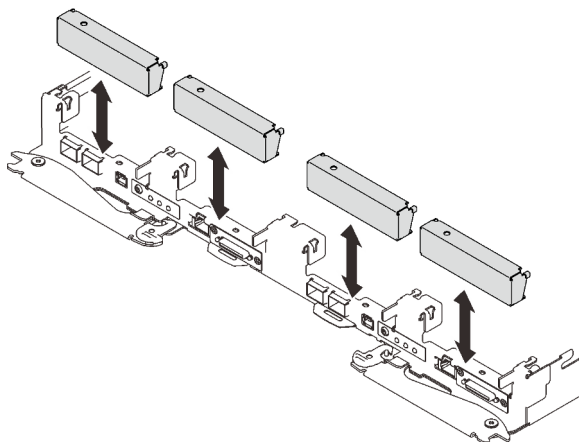
Figure 183. Installation de l'obturateur du panneau
