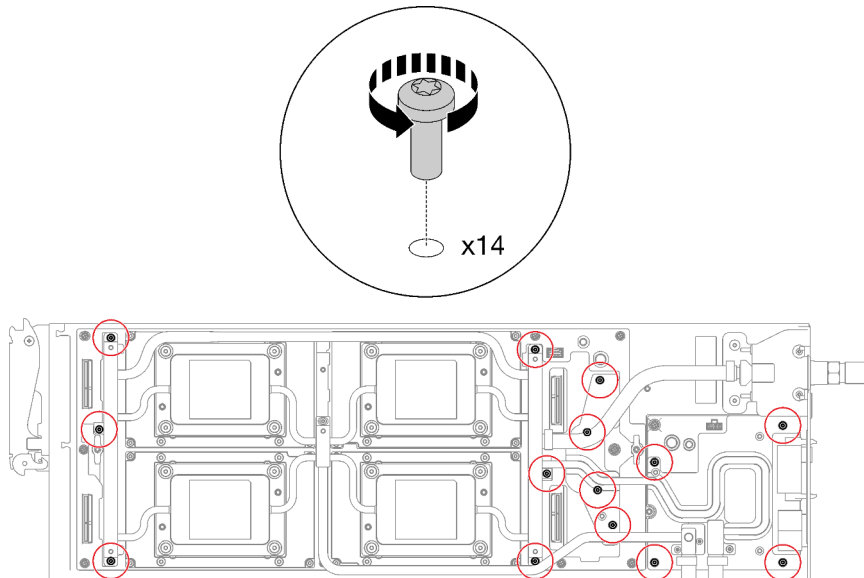
Figure 257. Retrait des vis de la boucle d'eau
