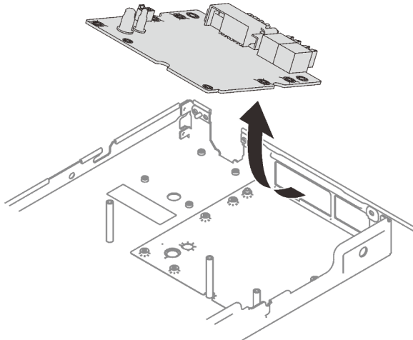
Figure 305. Retrait du tableau de distribution du GPU
