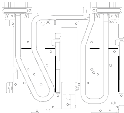
Figure 132. Marquages sur la boucle d'eau pour aligner le tampon d'espace E3.S
