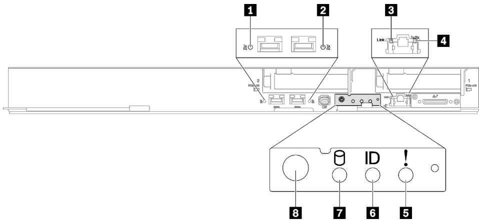
Figure 326. Voyants avant du plateau SD650-I V3
