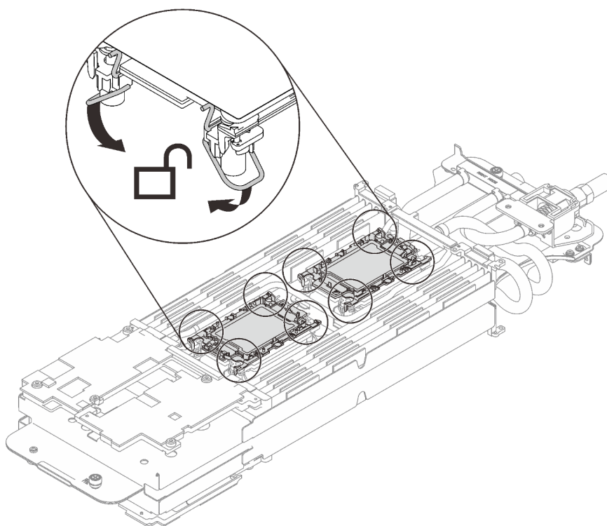
Figure 48. Position déverrouillée du processeur
