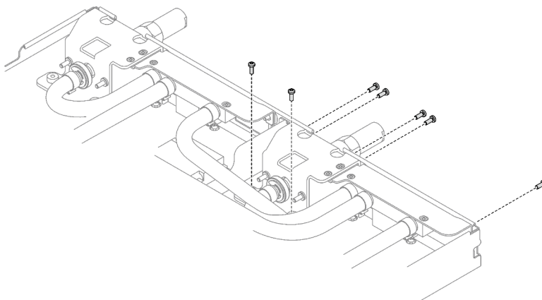
Figure 245. Installation des vis du raccord rapide
