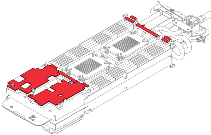
Figure 212. Tampons d'espace de la boucle d'eau
