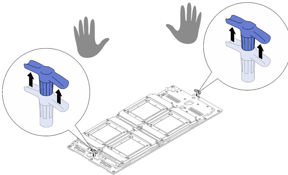
Figure 280. Retrait de la carte de base du support de la boîte d'emballage
