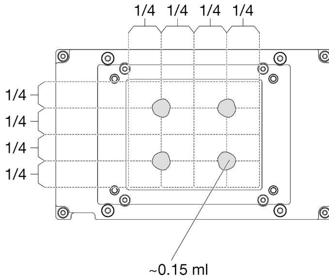
Figure 54. Application de la pâte thermoconductrice
