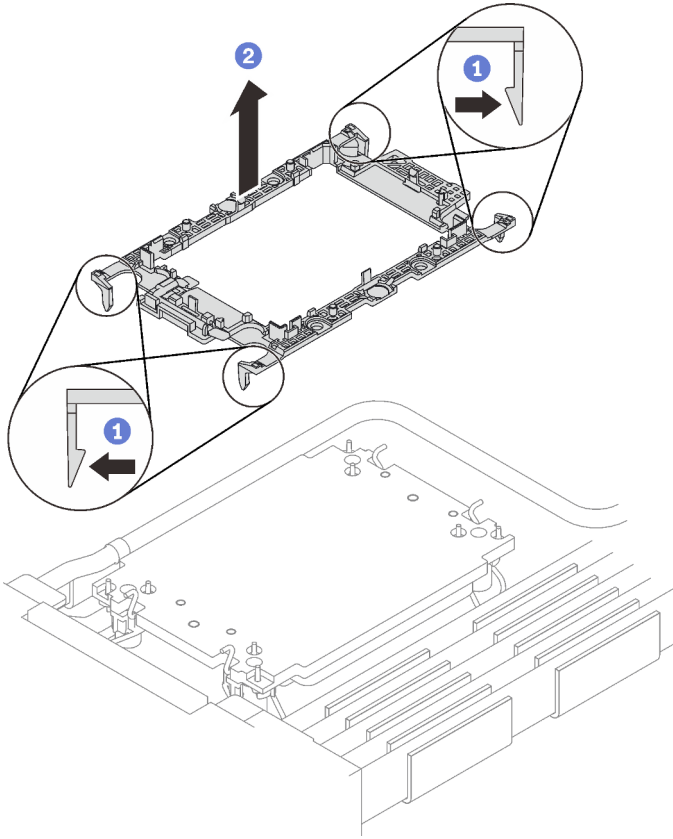
Figure 230. Retrait du dispositif de retenue du processeur
