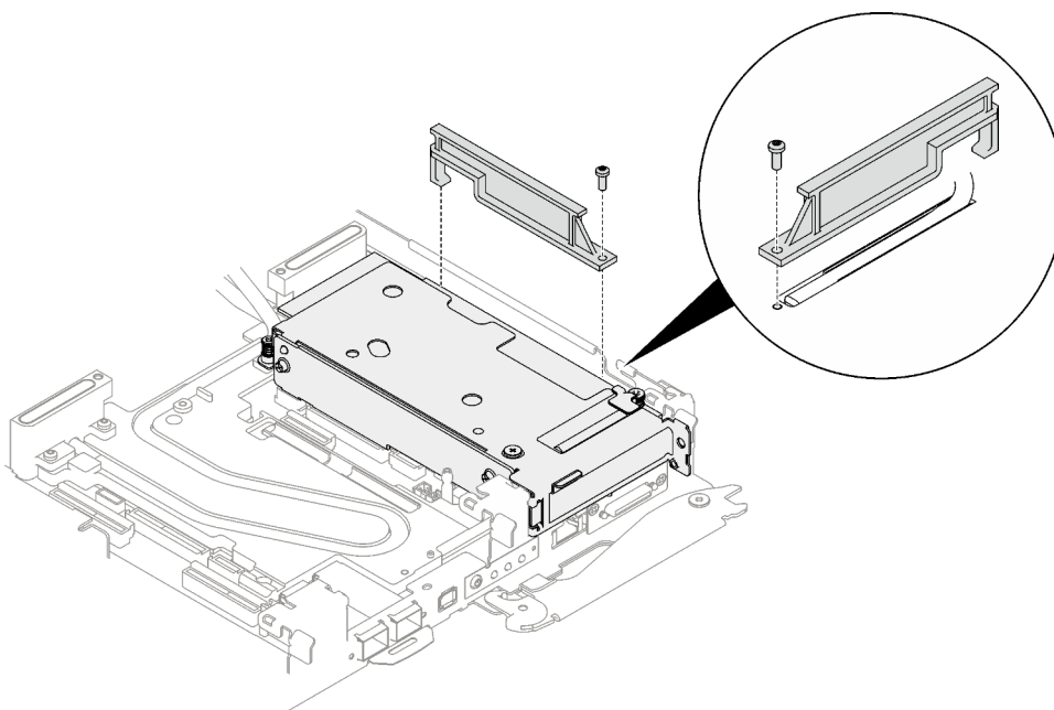
Figure 176. Installation du profilé du tube thermique
