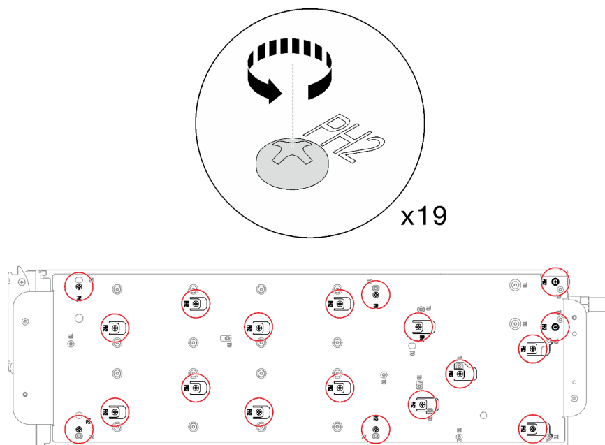
Figure 313. Desserrage des vis du support de la boucle d'eau
