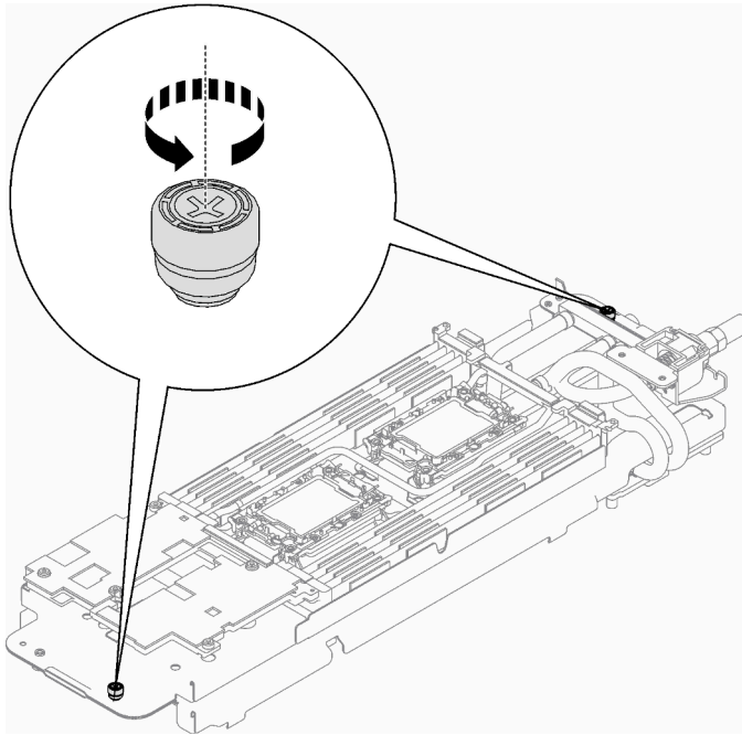
Figure 52. Desserrement des vis moletées imperdables
