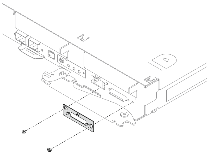
Figure 136. Retrait du cache KVM
