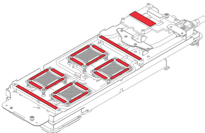
Figure 311. Emplacements des tampons de mastic
