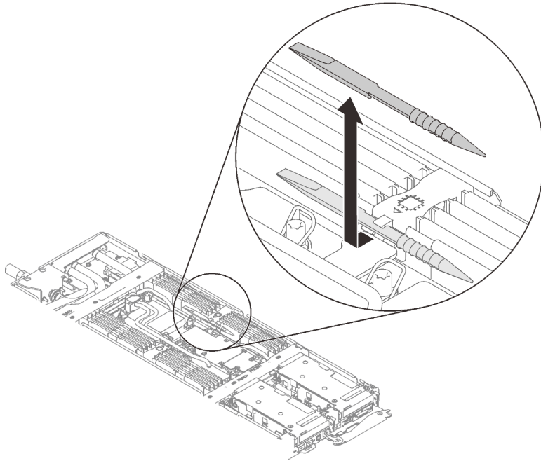
Figure 71. Retrait de l'outil du module de mémoire
