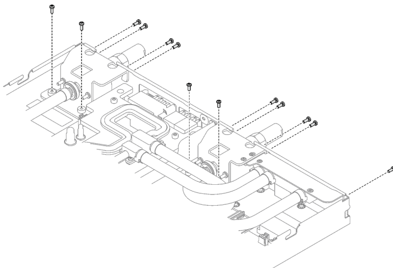
Figure 62. Installation des vis du raccord rapide
