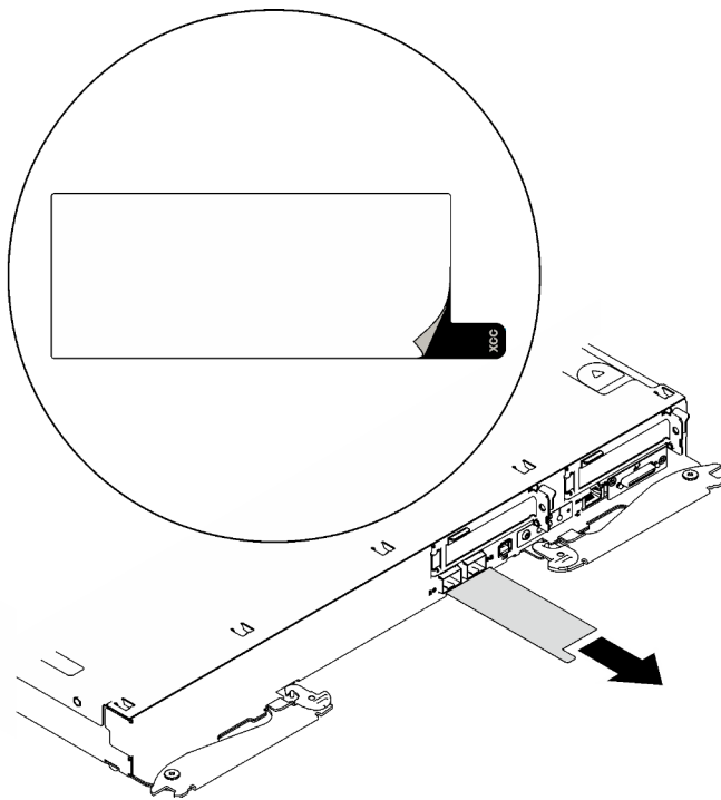
Figure 14. Étiquette d'accès réseau Lenovo XClarity Controller figurant sur l'étiquette amovible
