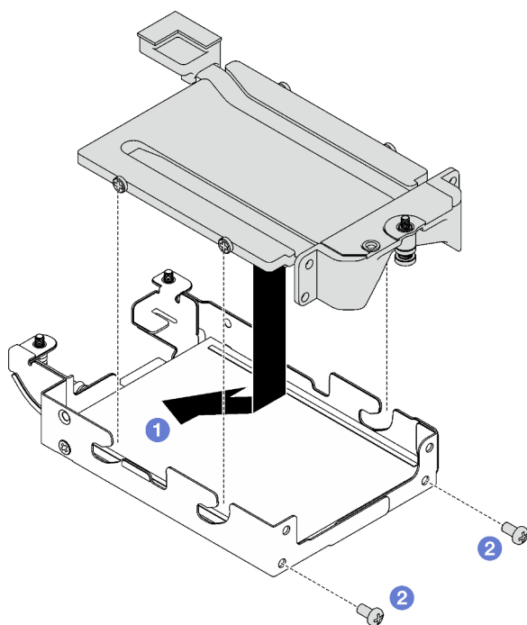
Figure 126. Installation de la plaque de conduction d'unité E3.s
