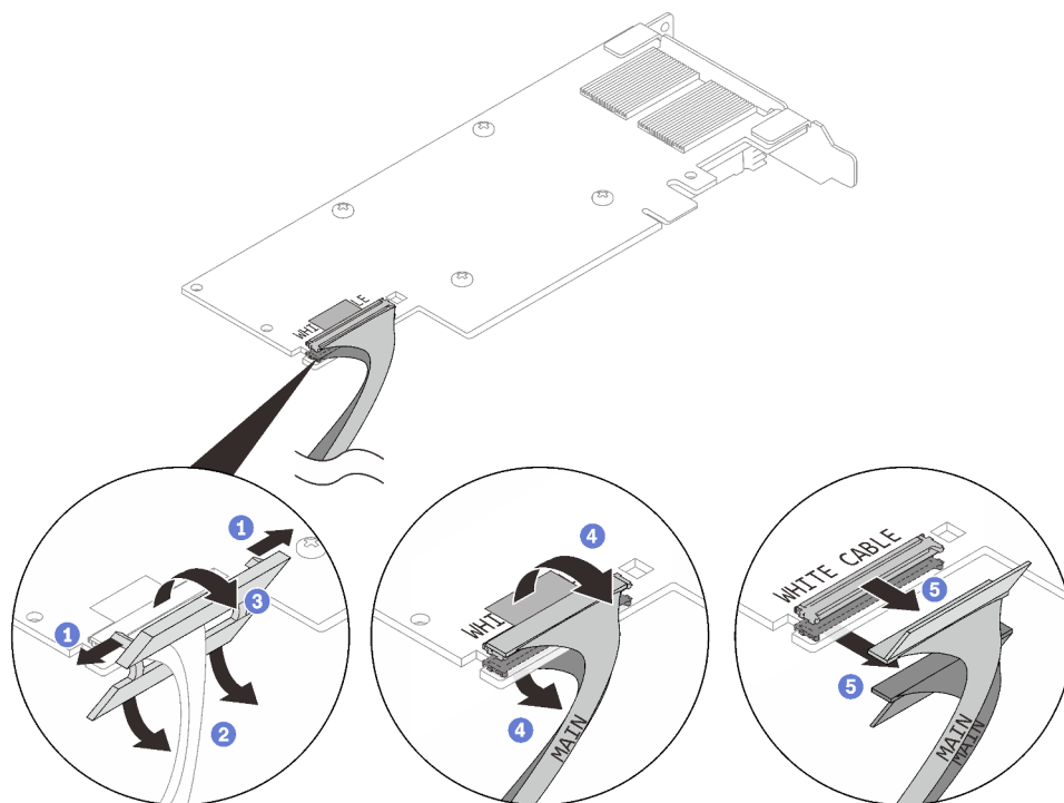
Figure 160. Retrait d'un câble d'adaptateur PCIe
