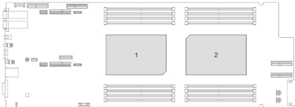
Figure 231. Emplacements des processeurs
