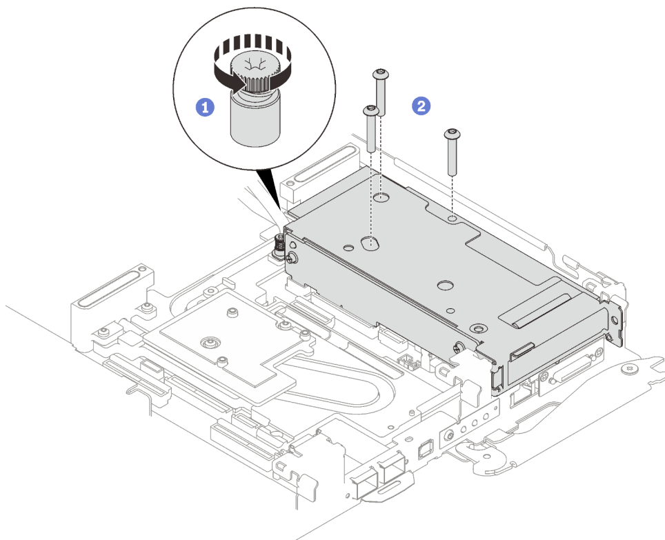
Figure 190. Retrait de l'assemblage de cartes mezzanines PCIe
