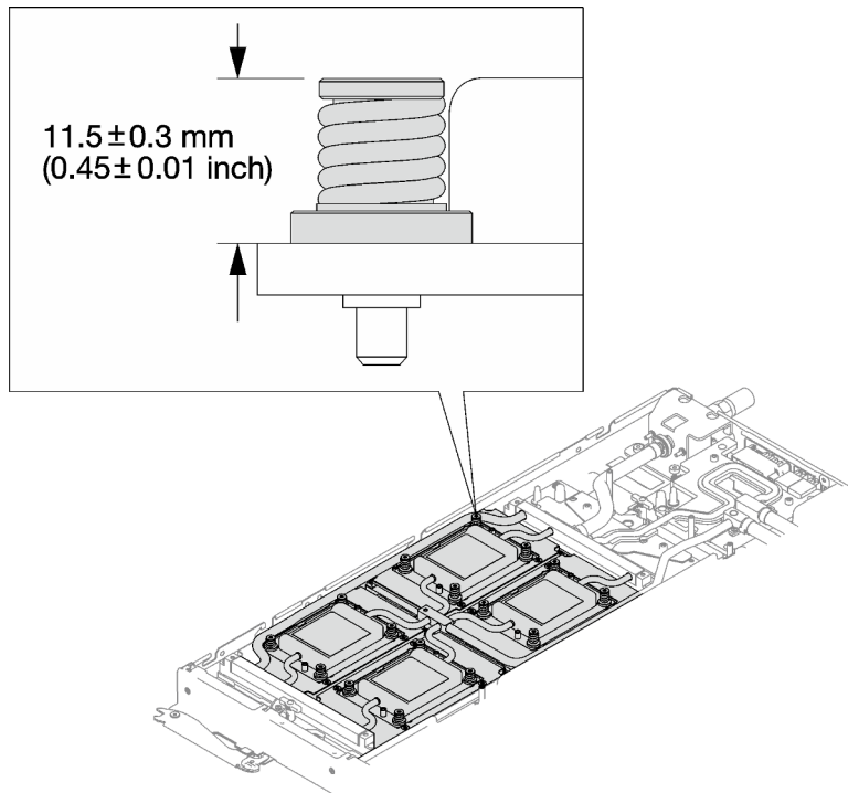
Figure 277. Hauteur de la vis de la plaque froide du GPU OAM correctement installée
