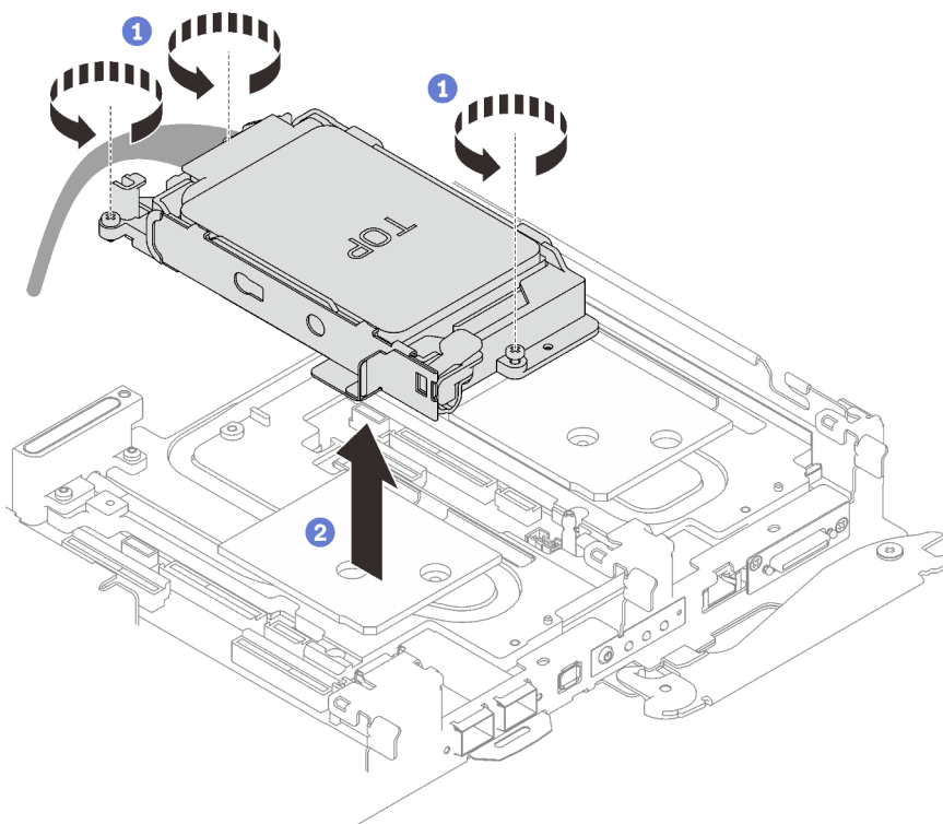
Figure 78. Retrait de deux blocs boîtiers d'unités de disque dur 7 mm
