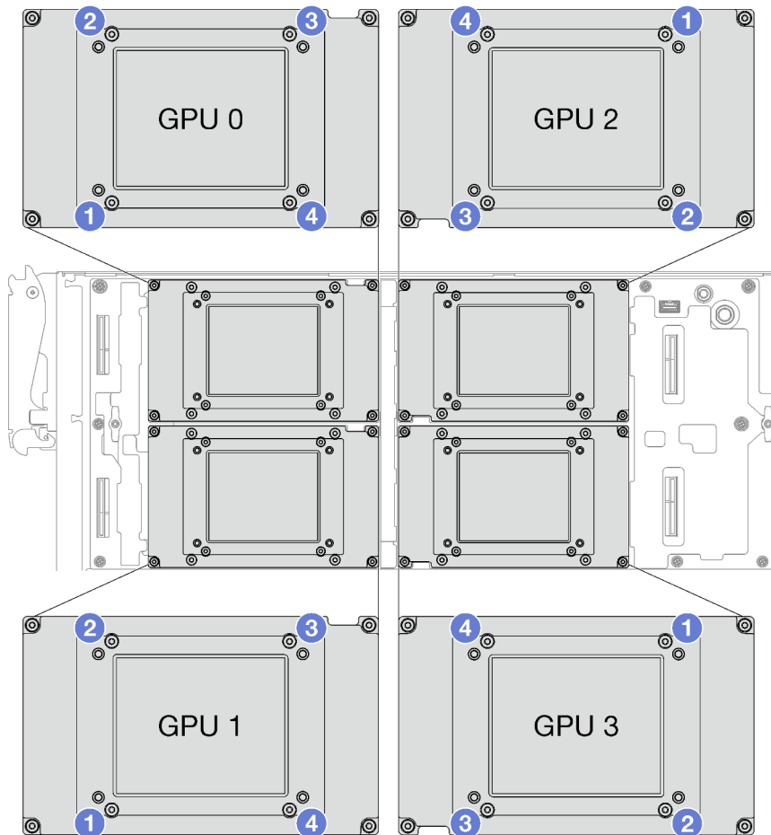
Figure 266. Séquence de serrage des vis pour l'installation du GPU OAM
