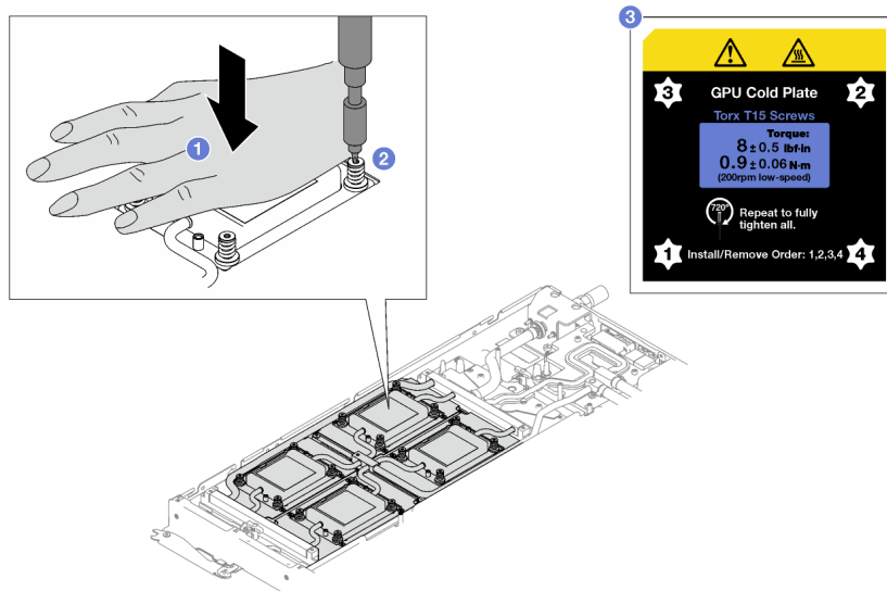
Figure 293. Serrage des vis de la plaque froide du GPU OAM sur 720 degrés
