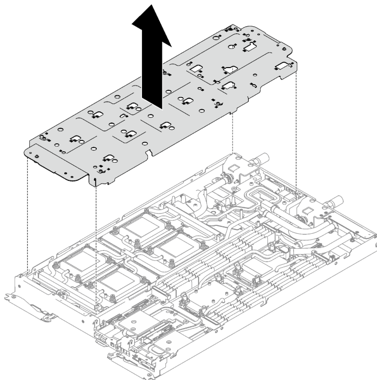
Figure 314. Retrait du support de la boucle d'eau
