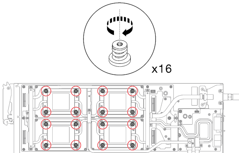
Figure 292. Installation des vis de la plaque froide du GPU OAM
