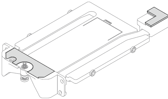
Figure 125. Remplacement des tampons de mastic de la plaque de conduction
