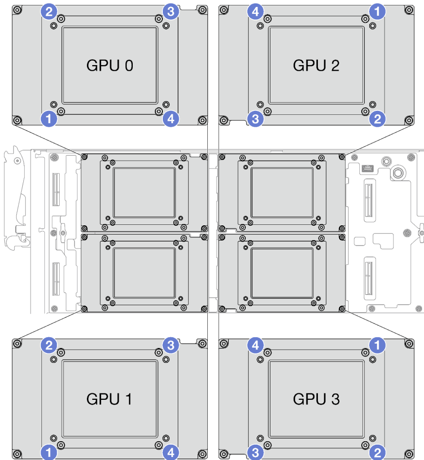
Figure 283. Séquence de serrage des vis pour l'installation du GPU OAM
