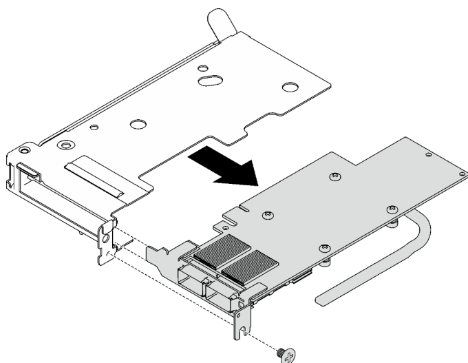
Figure 159. Retrait d'un adaptateur PCIe
