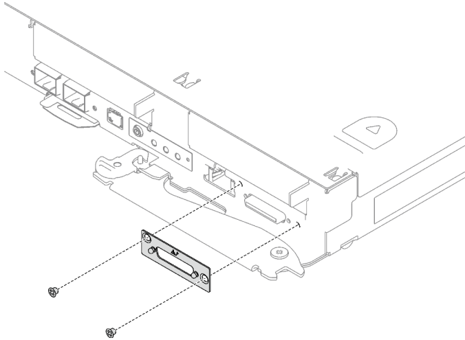
Figure 137. Installation d'un cache KVM
