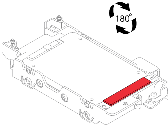
Figure 91. Emplacement du tampon d'espace
