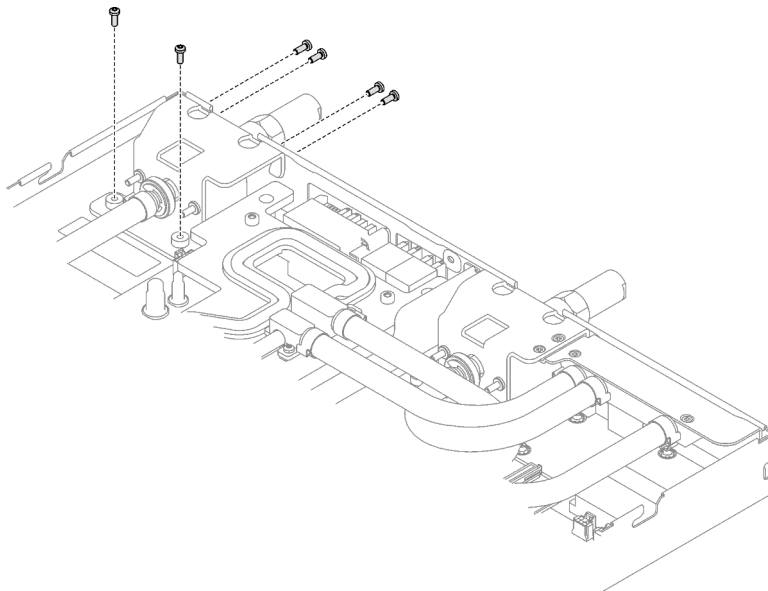
Figure 256. Retrait des vis du raccord rapide
