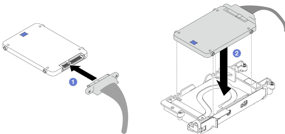
Figure 106. Installation de l'unité inférieure
