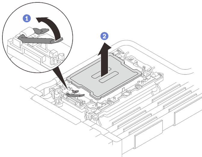
Figure 228. Retrait d'un processeur
