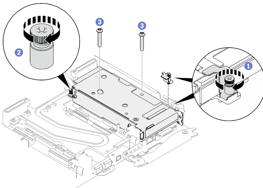
Figure 189. Installation de la vis imperdable de l'étrier de fixation
