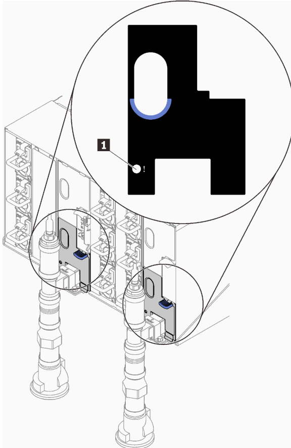
Figure 330. Voyant du capteur de gouttes
