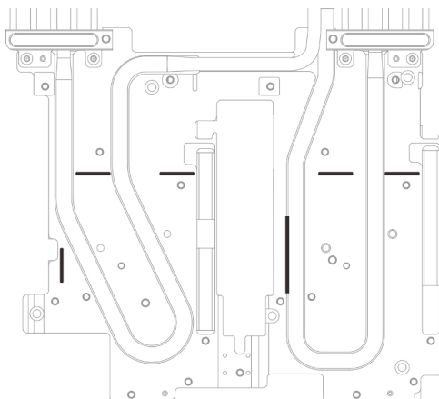
Figure 109. Marquages sur la boucle d'eau pour aligner le tampon d'espace
