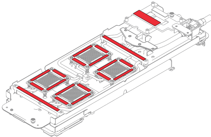
Figure 51. Emplacements des tampons de mastic
