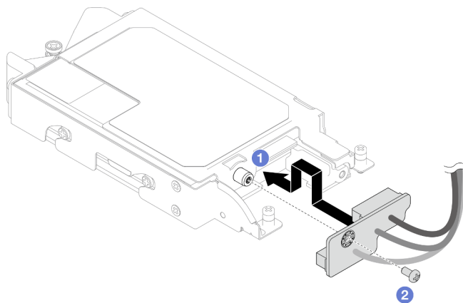
Figure 128. Installation d'un fond de panier doté d'un câble d'unité E3.s à son extrémité
