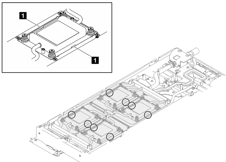
Figure 30. Encoches sur la plaque froide du GPU OAM
