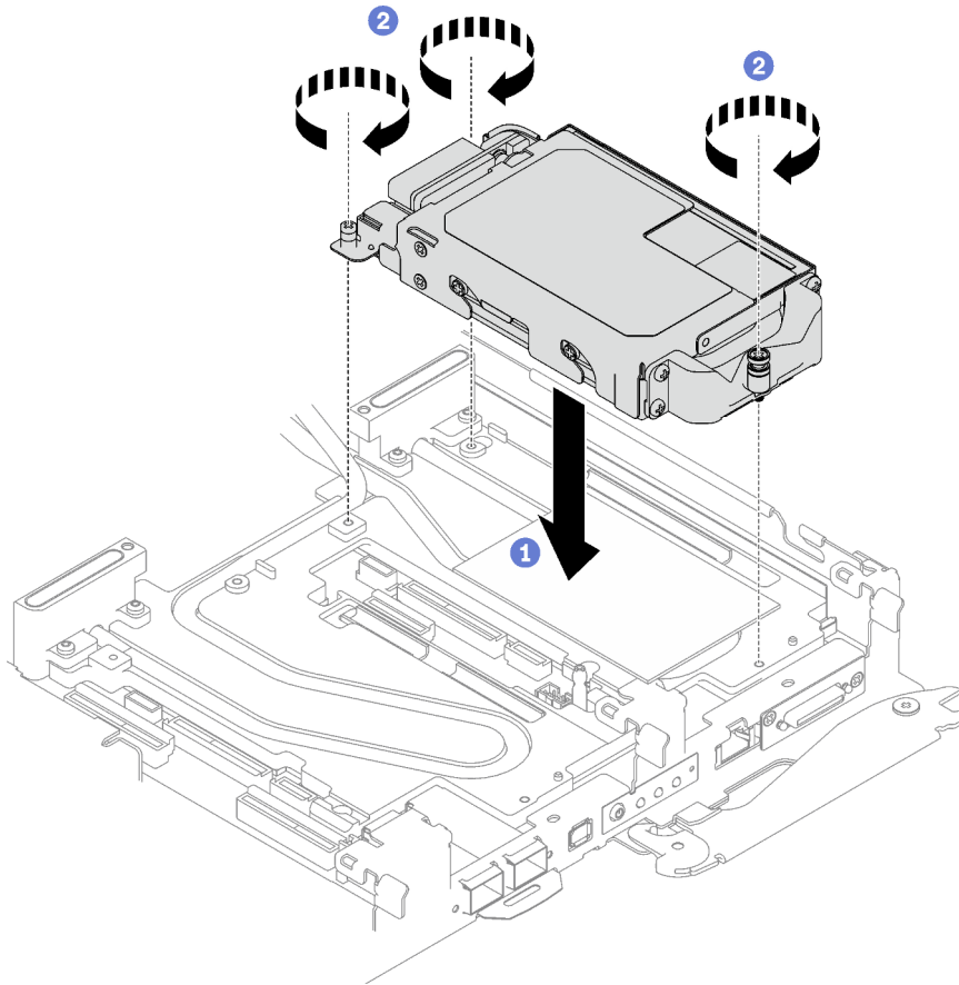
Figure 134. Installation du bloc boîtier d'unités de disque dur E3.S
