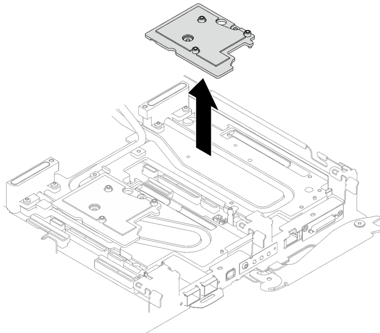
Figure 196. Retrait de la plaque d'interface
