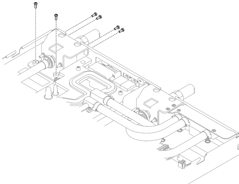
Figure 291. Installation des vis du raccord rapide
