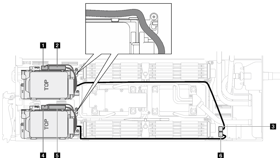
Figure 114. Cheminement des câbles du bloc unité
