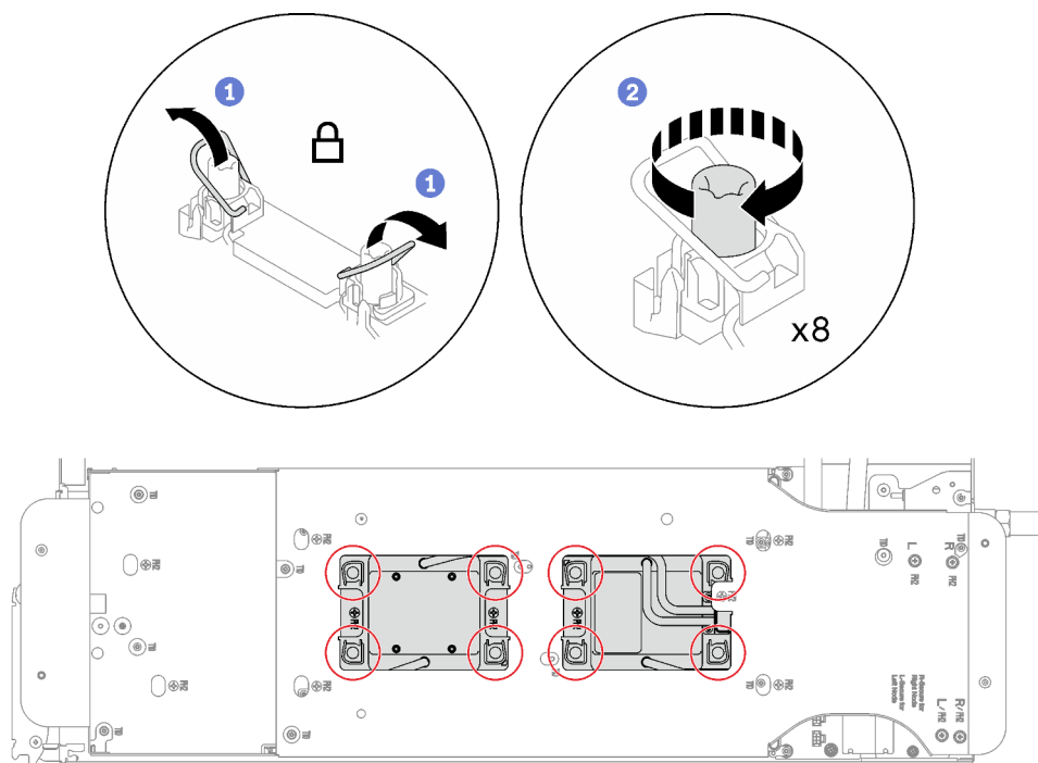
Figure 241. Installation des processeurs
