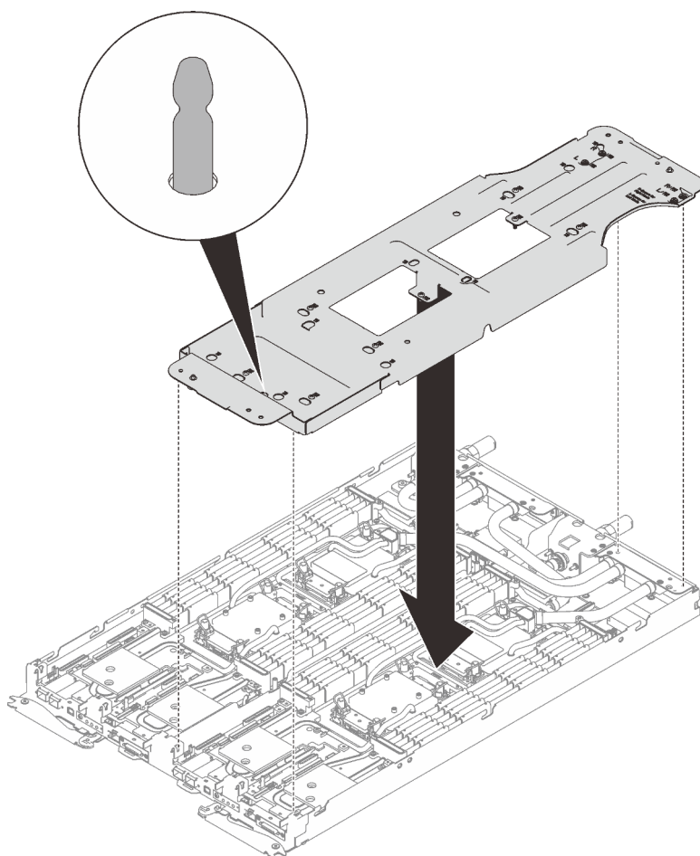
Figure 206. Installation du support de boucle d'eau
