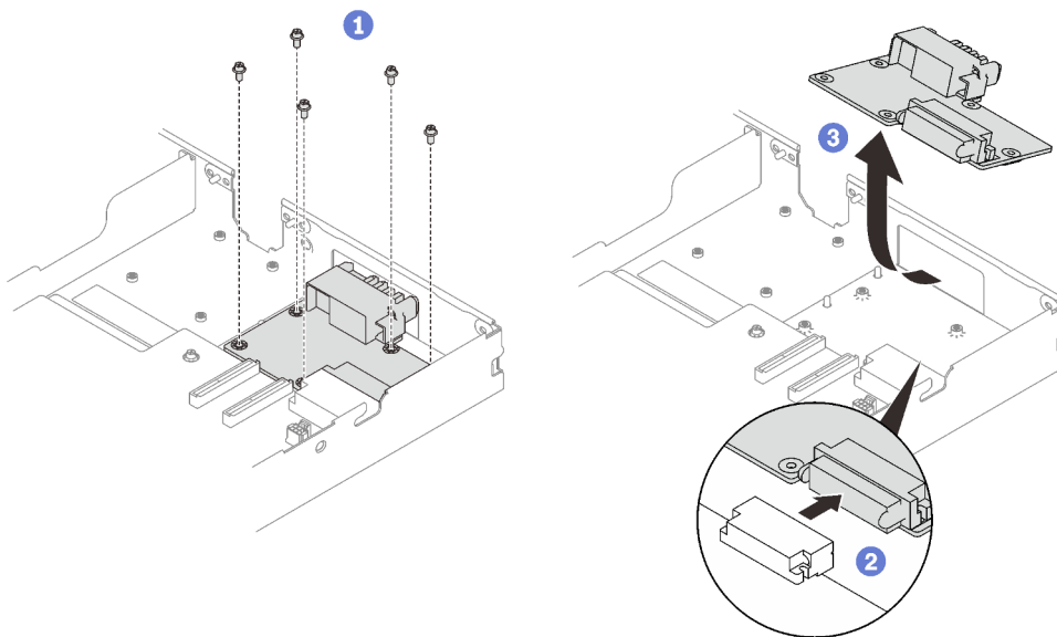
Figure 210. Tableau de distribution, retrait
