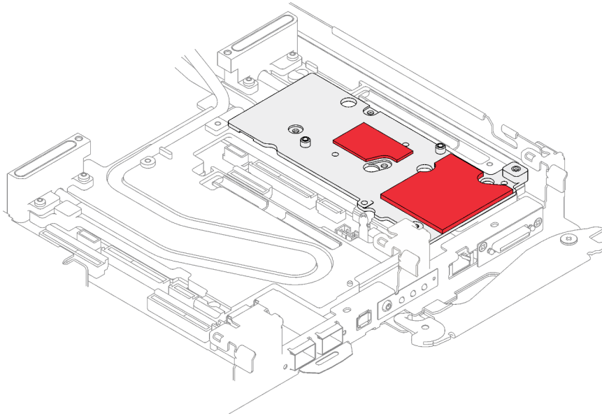
Figure 187. Plaque d'interface sur plaque froide pour CX-7 NDR 200
