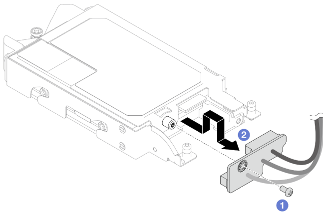
Figure 119. Retrait du fond de panier doté d'un câble d'unité E3.S à son extrémité
