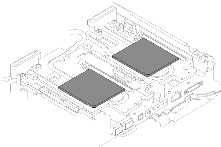
Figure 111. Emplacements des tampons d'espace
