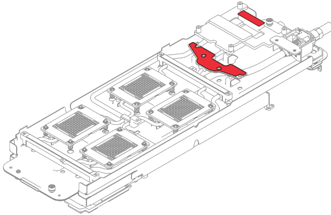
Figure 50. Emplacements des tampons d'espace
