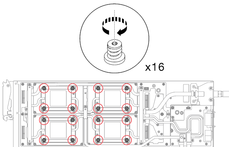
Figure 63. Installation des vis de la plaque froide du GPU OAM
