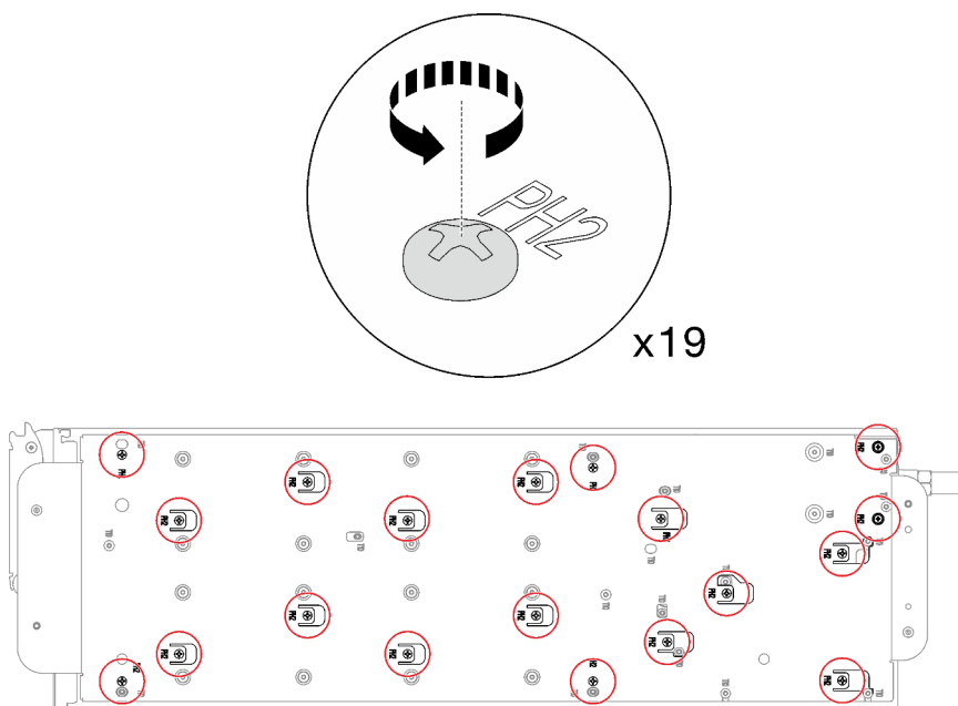
Figure 271. Desserrage des vis du support de la boucle d'eau
