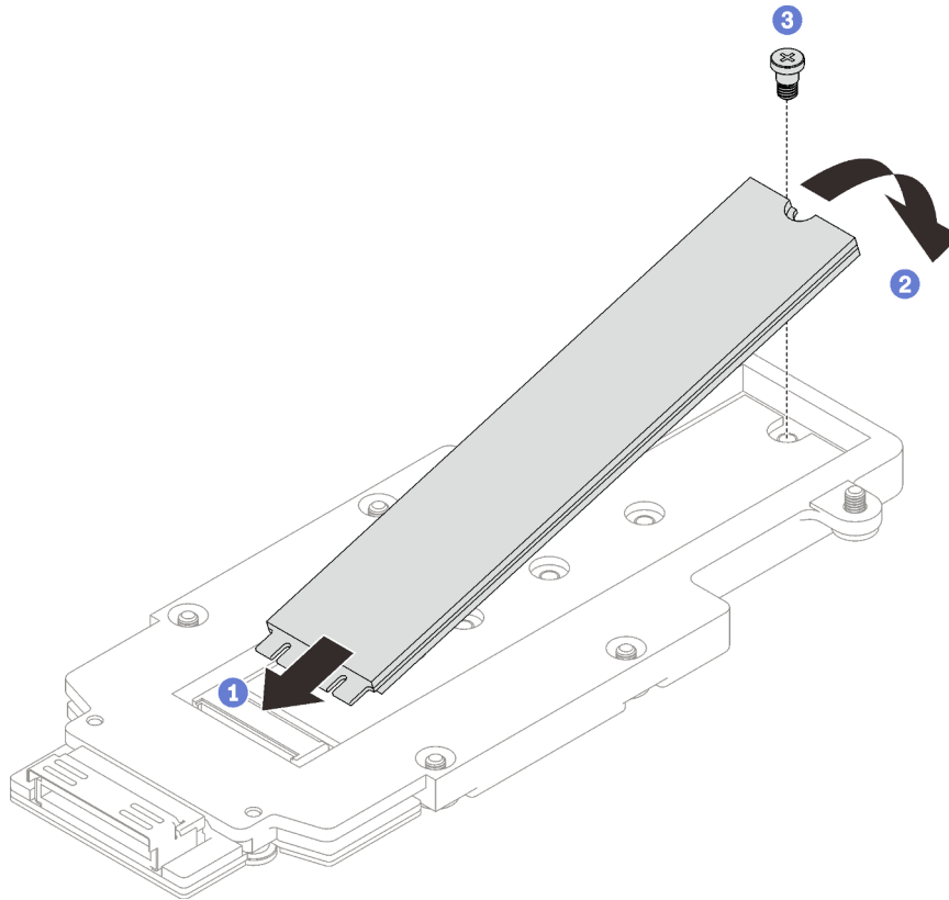
Figure 144. Installation d'une unité M.2
