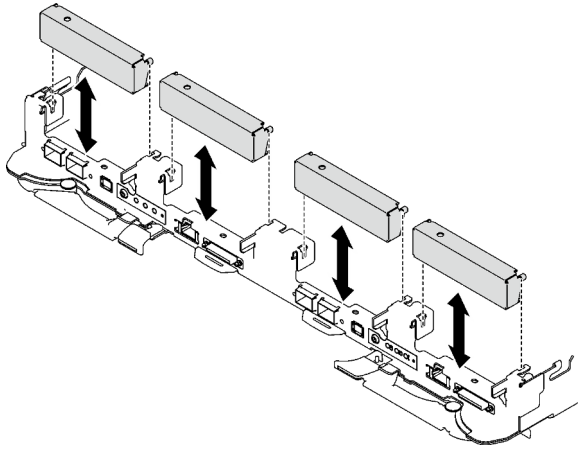
Figure 101. Retrait de l'obturateur vide du panneau
