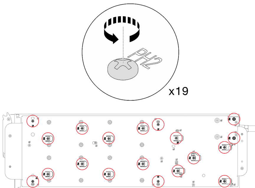
Figure 288. Desserrage des vis du support de la boucle d'eau
