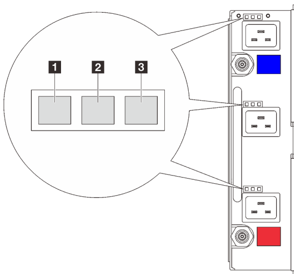
Figure 329. Voyants de l'alimentation DWC
