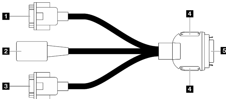
Figure 5. Connecteurs et composants sur le câble d'interface KVM
