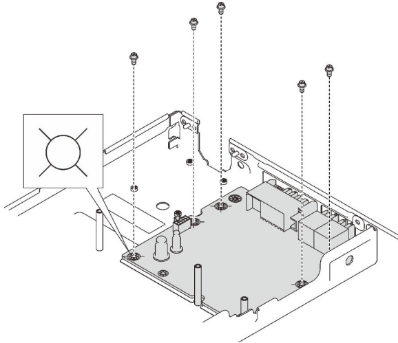
Figure 304. Retrait des vis
