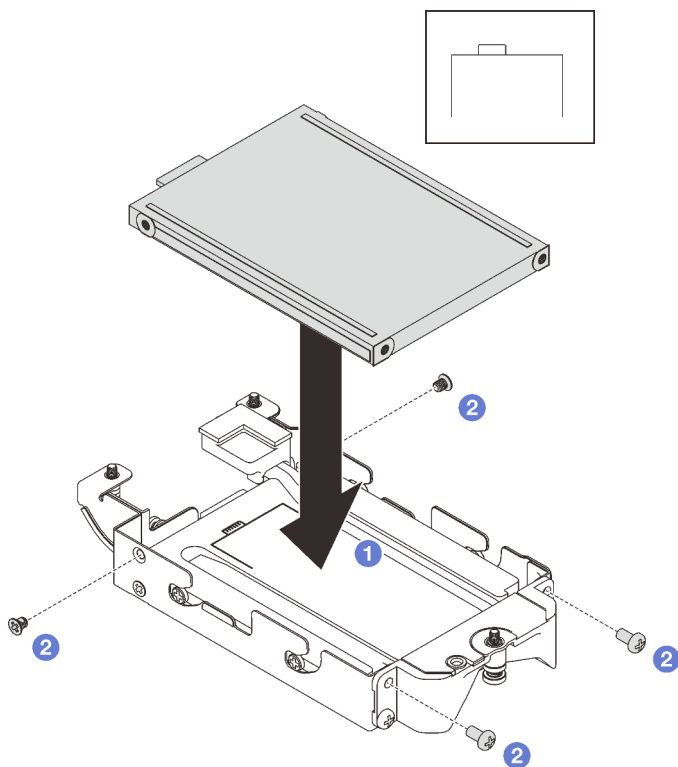
Figure 127. Installation de l'unité E3.s inférieure
