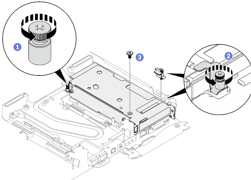
Figure 166. Retrait de la vis imperdable de l'étrier de fixation
