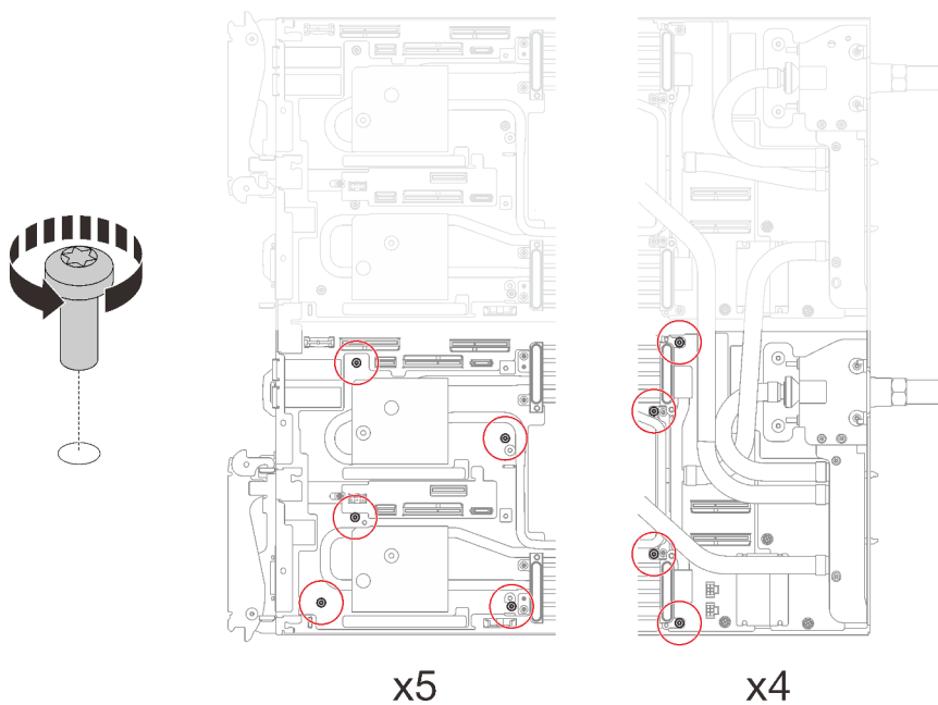
Figure 222. Retrait des vis de la boucle d'eau
