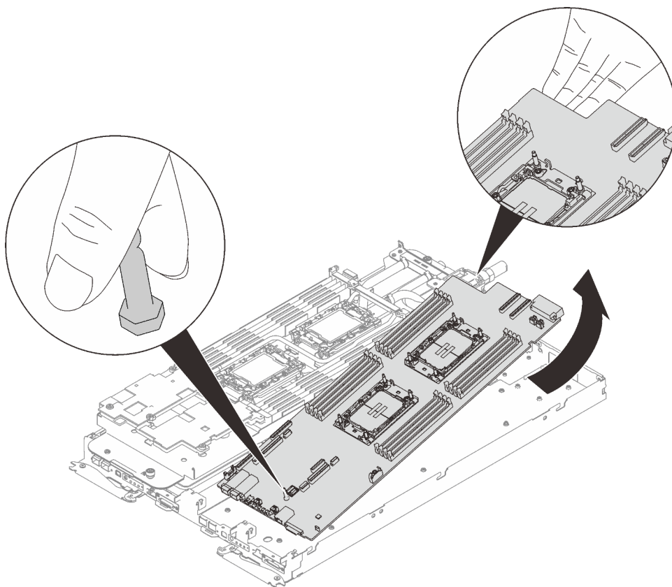
Figure 249. Retrait de la carte mère
