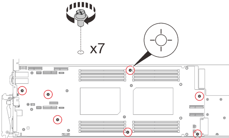
Figure 248. Retrait des vis de la carte mère
