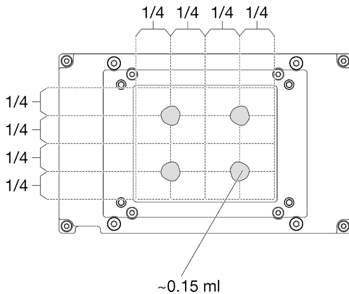
Figure 284. Application de la pâte thermoconductrice
