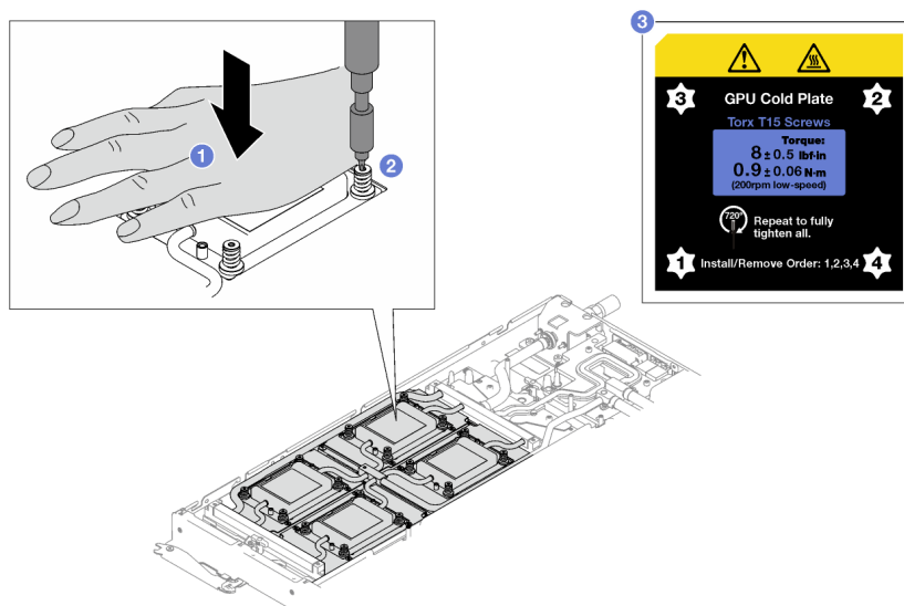
Figure 64. Serrage des vis de la plaque froide du GPU OAM sur 720 degrés
