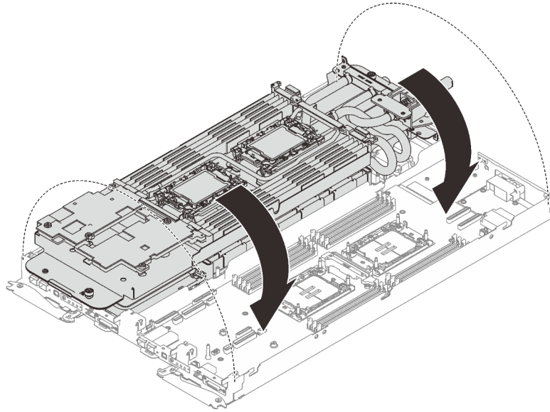
Figure 240. Installation de la boucle d'eau
