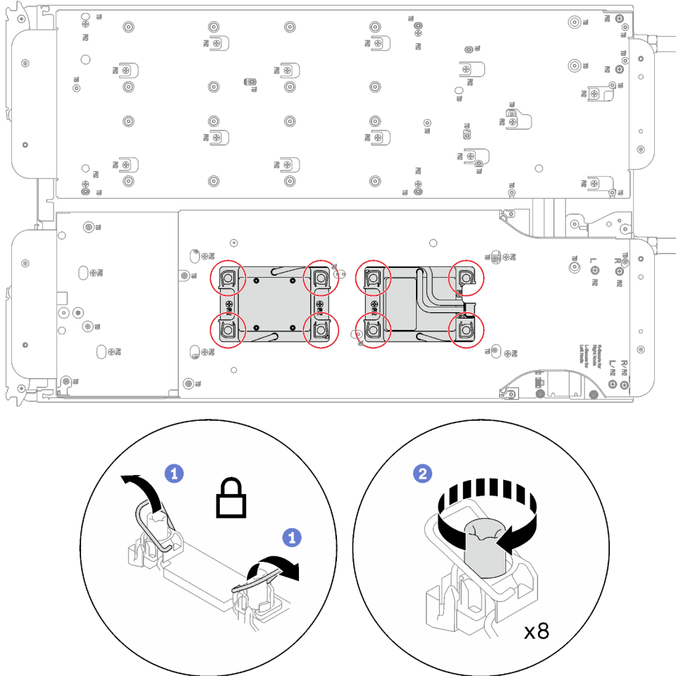
Figure 58. Serrage des vis imperdables Torx T30
