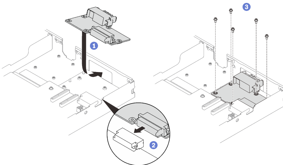
Figure 211. Installation du tableau de distribution
