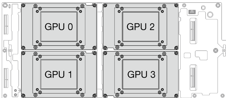
Figure 281. Numérotation du GPU OAM
