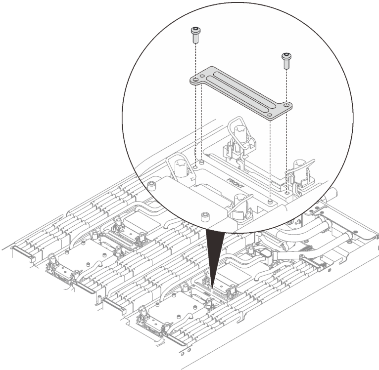
Figure 203. Retrait de la plaque de serrage VR
