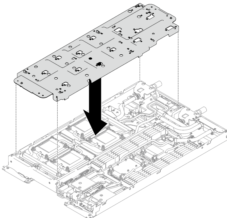
Figure 301. Installation du support de boucle d'eau
