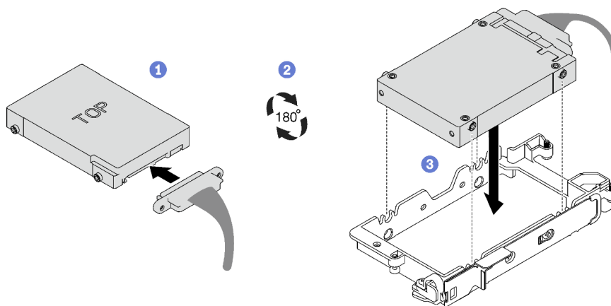
Figure 86. Installation de l'unité 15 mm
