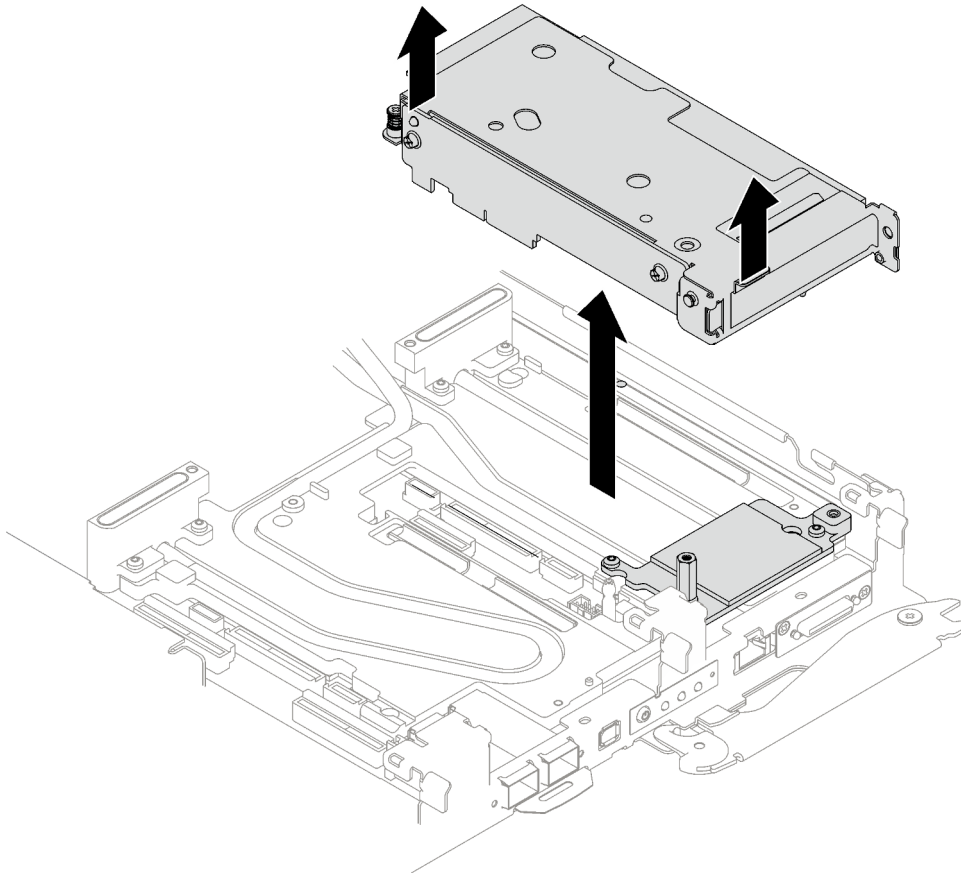
Figure 167. Retrait de l'assemblage de cartes mezzanines PCIe
