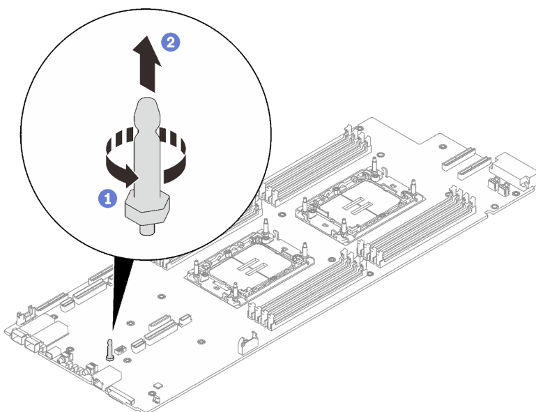
Figure 250. Retrait de la broche de guidage
