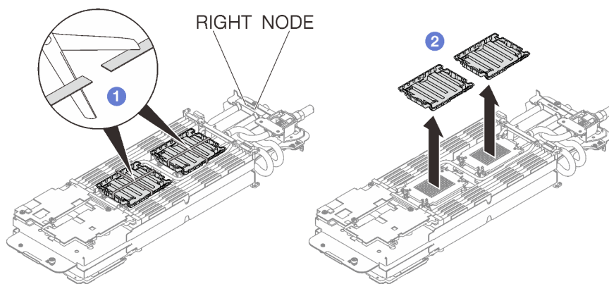
Figure 46. Retrait des films de protection en pâte thermoconductrice
