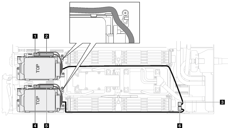
Figure 99. Cheminement des câbles du bloc unité
