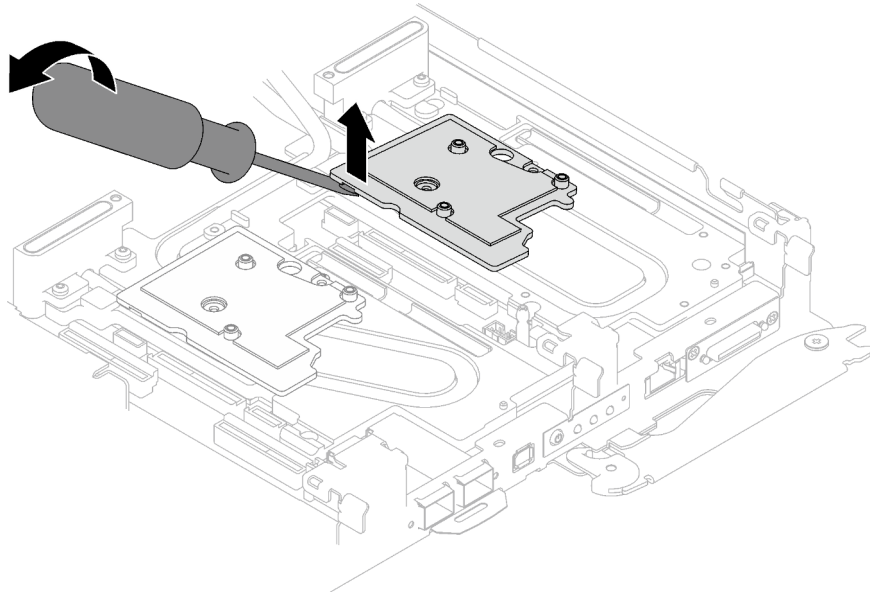
Figure 195. Libération de la plaque d'interface de la plaque froide de la boucle d'eau
