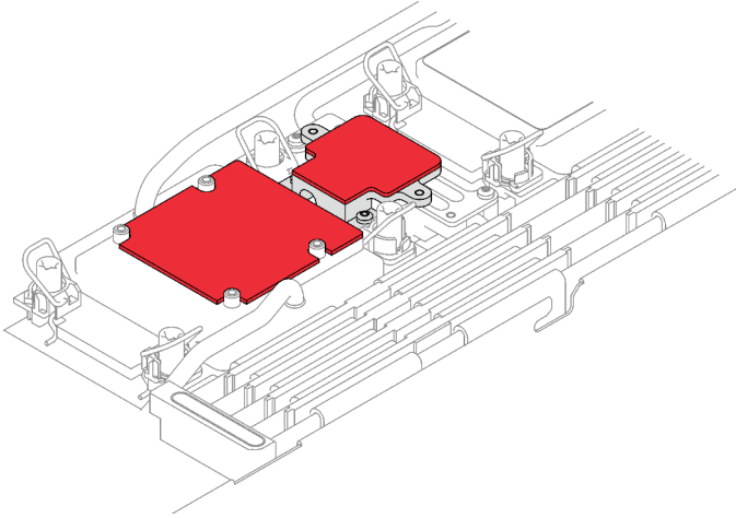
Figure 146. Tampon d'espacement sur la plaque froide du processeur et la plaque froide du fond de panier M.2
