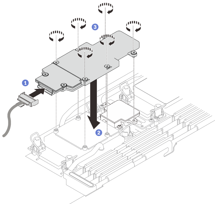
Figure 147. Installation du fond de panier M.2
