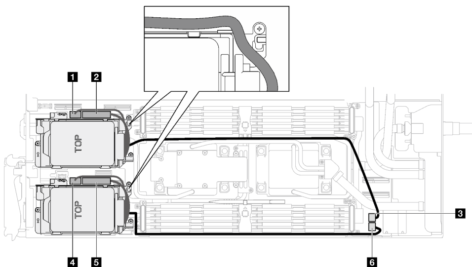
Figure 113. Cheminement des câbles du bloc unité
