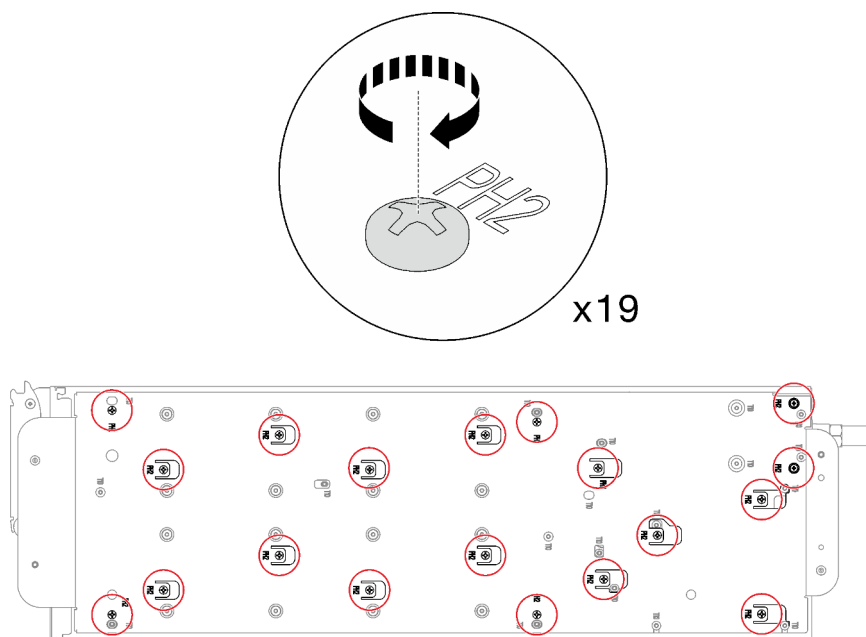
Figure 302. Installation des vis du support de boucle d'eau
