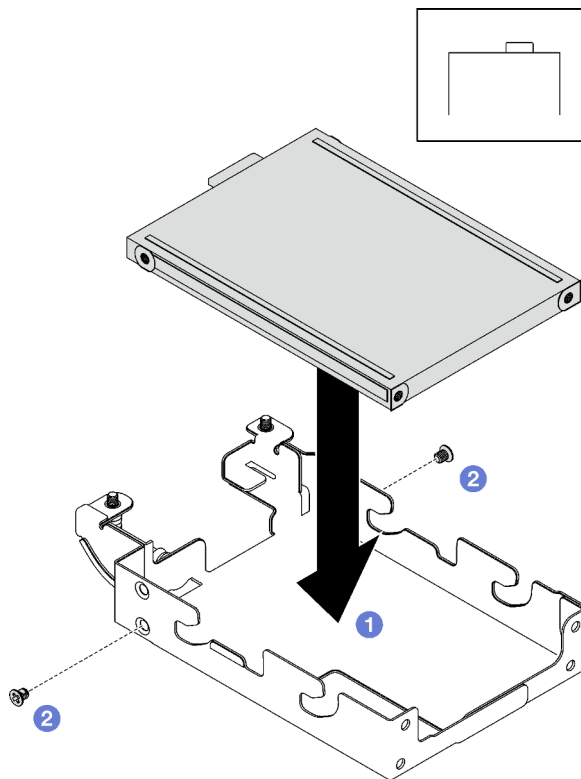
Figure 123. Installation de l'unité E3.S supérieure
