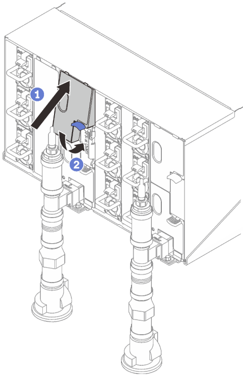
Figure 335. Installation du blindage EMC supérieur
