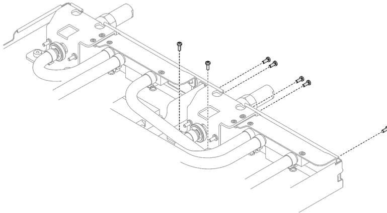
Figure 205. Retrait des vis du raccord rapide
