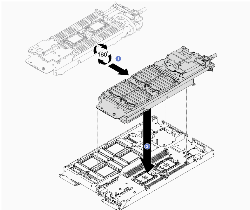
Figure 53. Installation du support de boucle d'eau
