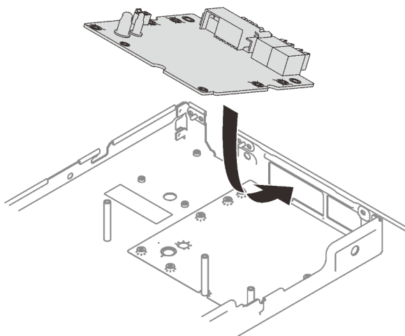
Figure 307. Installation du tableau de distribution du GPU
