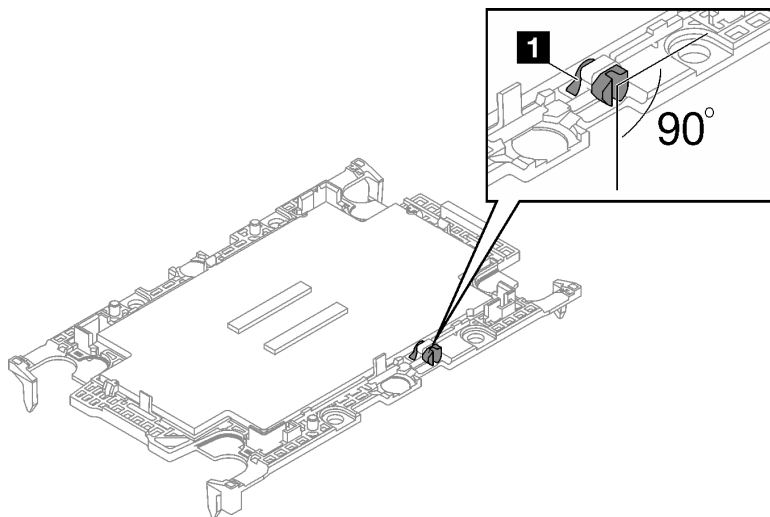
Figure 44. Came de rupture TIM sur le dispositif de retenue du processeur
