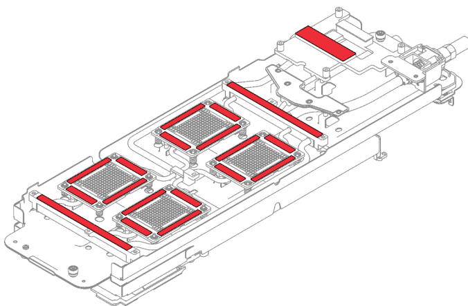
Figure 286. Emplacements des tampons de mastic
