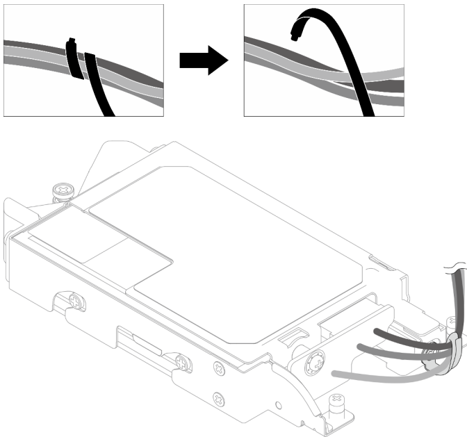
Figure 117. Dégagement des câbles de l'attache-câbles
