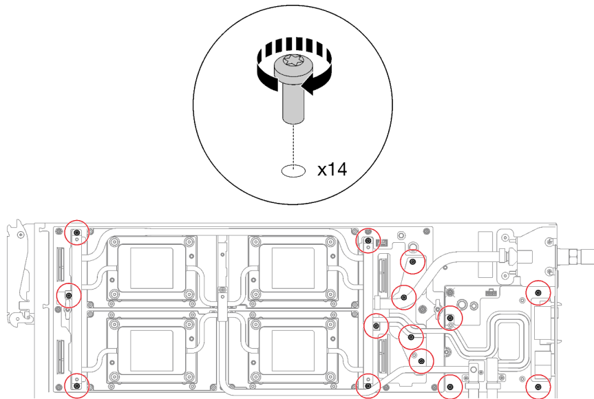
Figure 315. Installation des vis de la boucle d'eau
