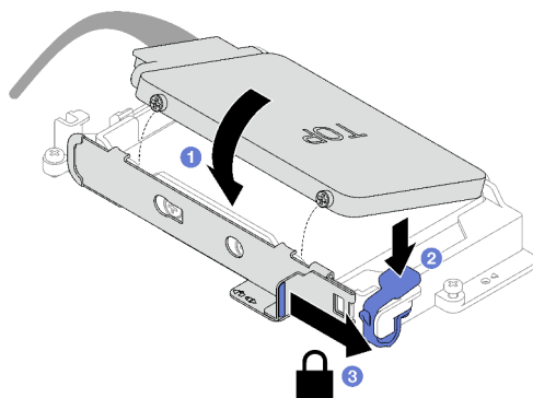
Figure 89. Installation de l'unité supérieure
