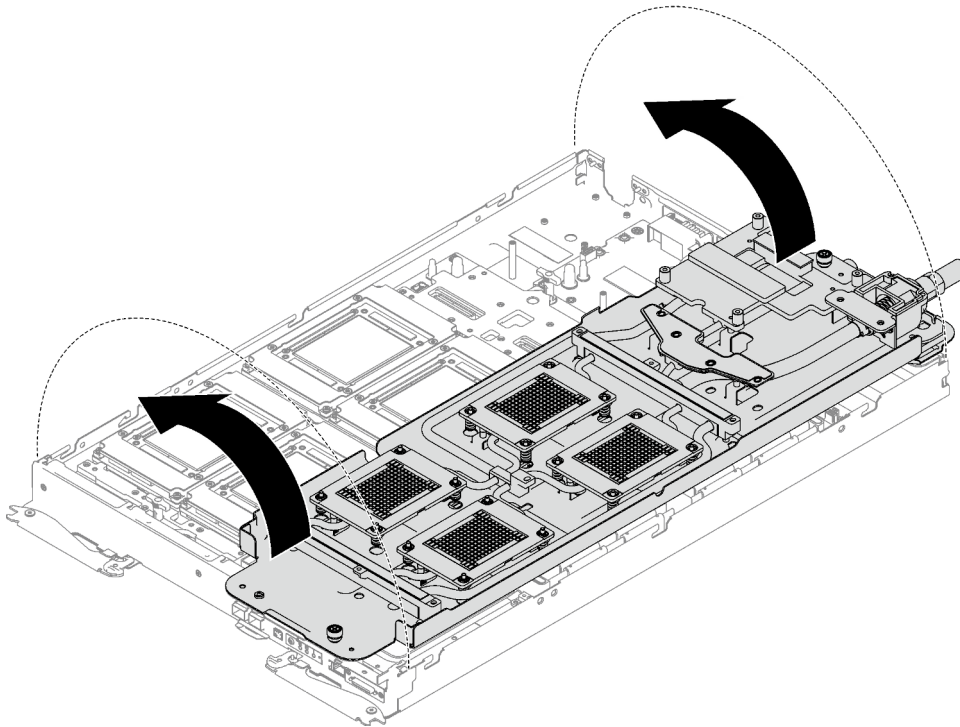
Figure 270. Installation de la boucle d'eau
