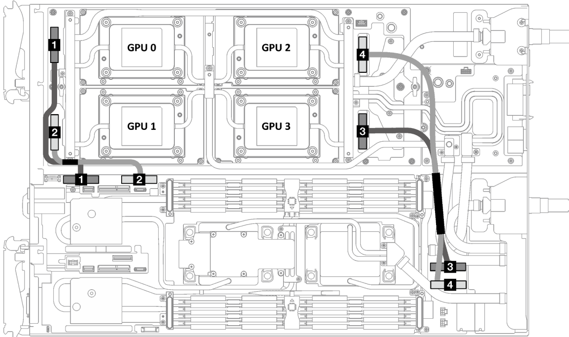
Figure 322. Cheminement des câbles de signal du plateau SD650-I V3
