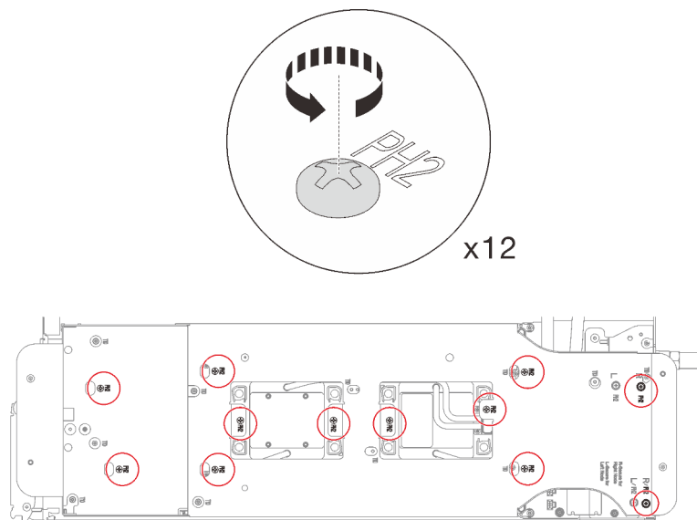
Figure 215. Desserrage des vis du support de la boucle d'eau
