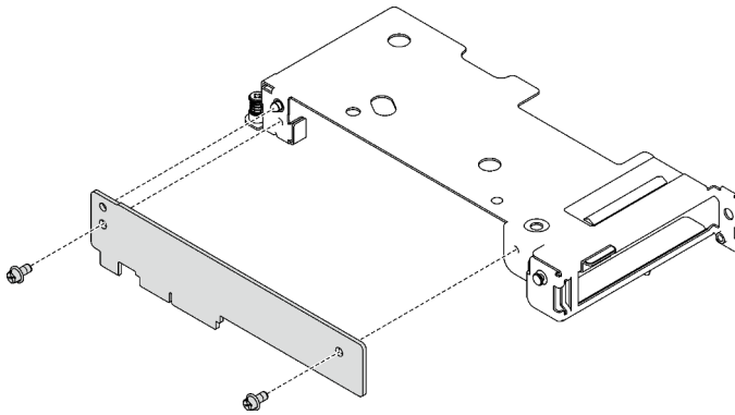
Figure 198. Retrait de la carte d'extension
