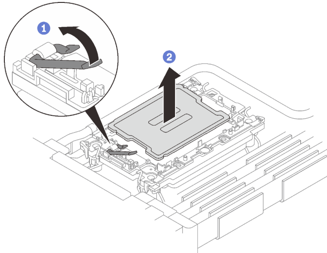
Figure 37. Retrait d'un processeur
