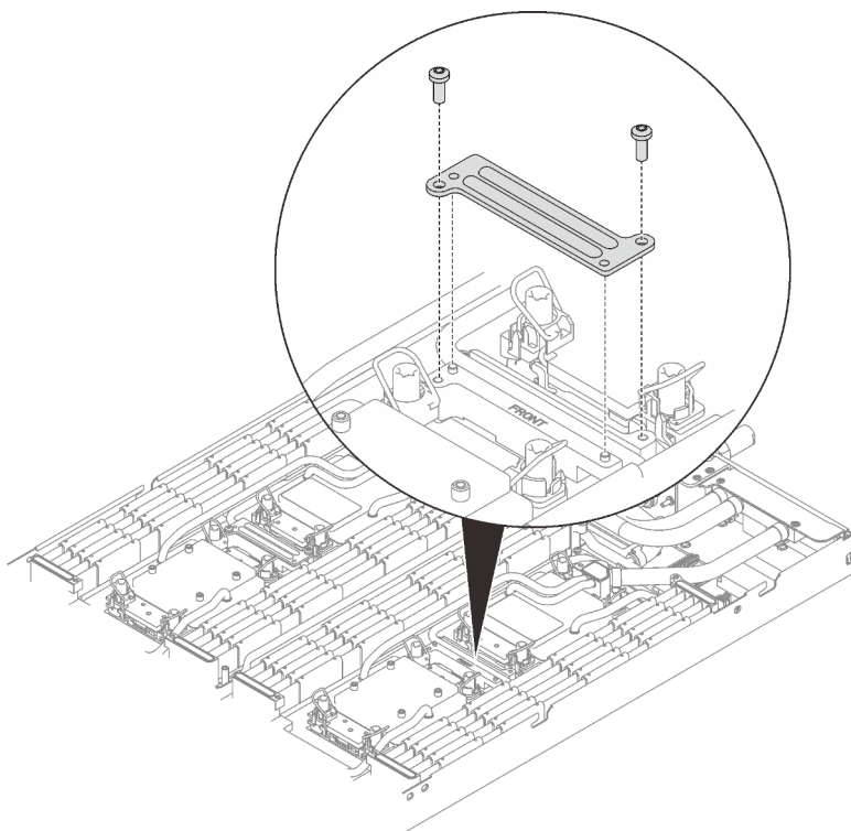
Figure 219. Installation de la plaque de serrage VR
