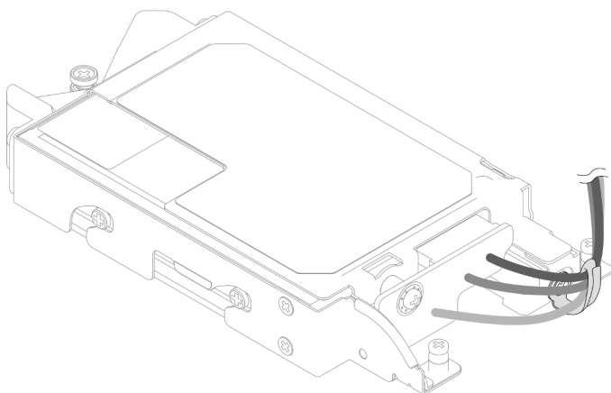
Figure 130. Groupement des câbles à l'aide d'un attache-câbles
