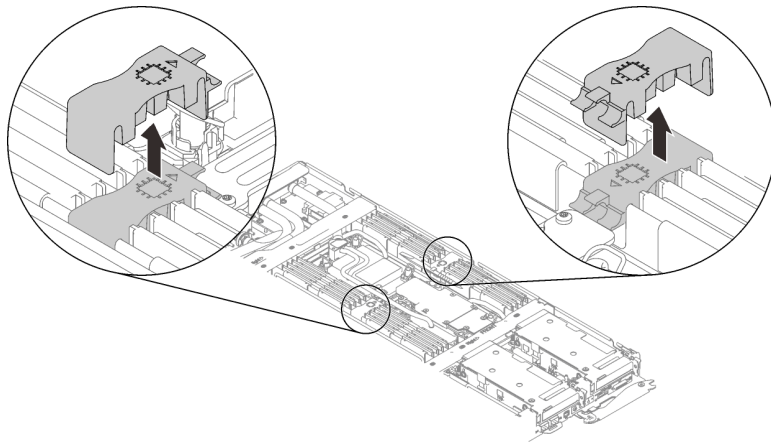
Figure 72. Retrait d'un ensemble DIMM
