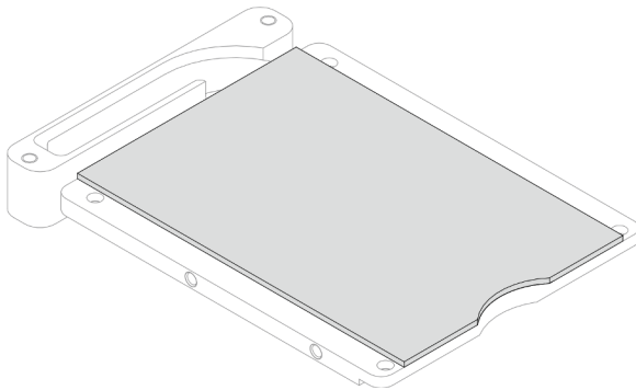
Figure 104. Installation d'une plaque de conduction dotée d'un tampon d'espace
