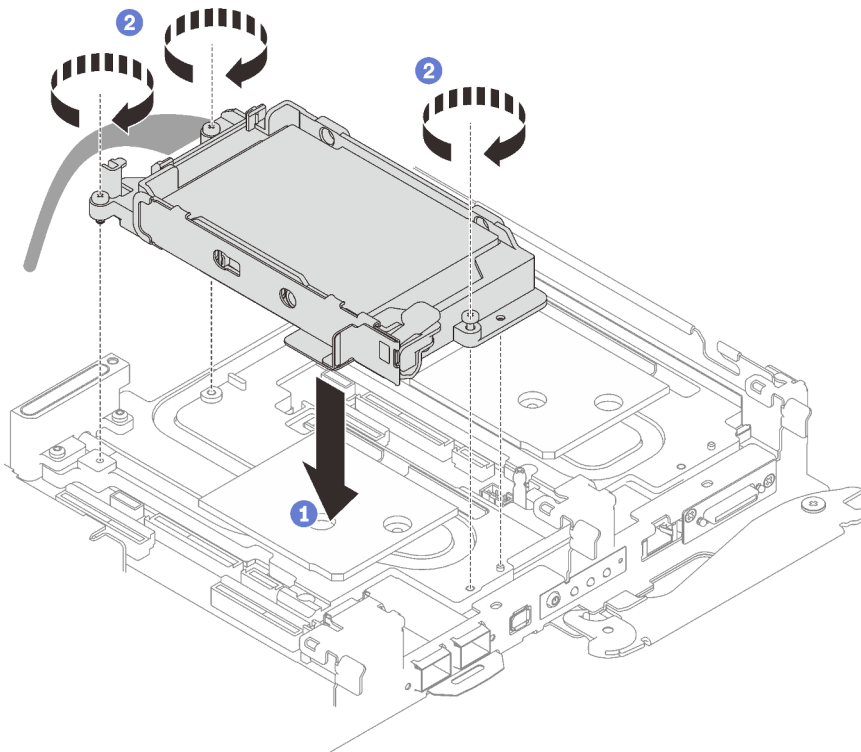
Figure 95. Installation d'un bloc boîtier d'unités de disque dur 15 mm
