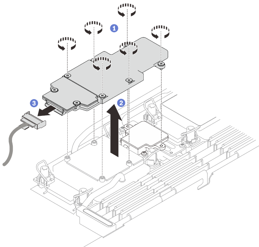
Figure 139. Retrait du fond de panier M.2
