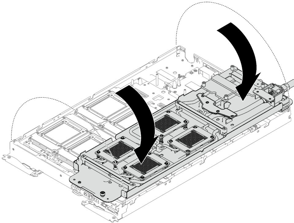
Figure 263. Plier la boucle d'eau
