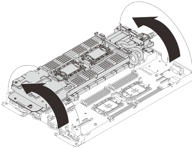
Figure 209. Plier la boucle d'eau
