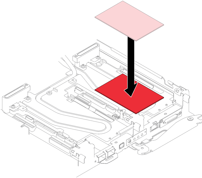
Figure 133. Remplacement du tampon d'espace
