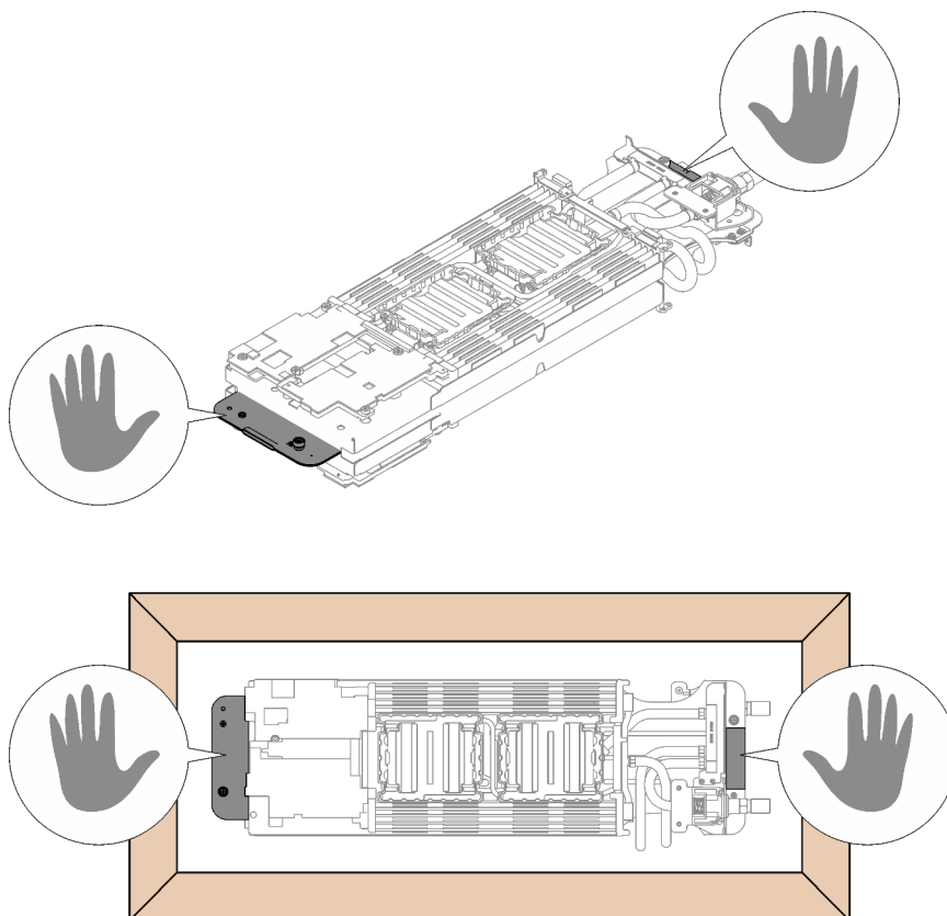
Figure 45. Points de contact lors du déballage de la boucle d'eau
