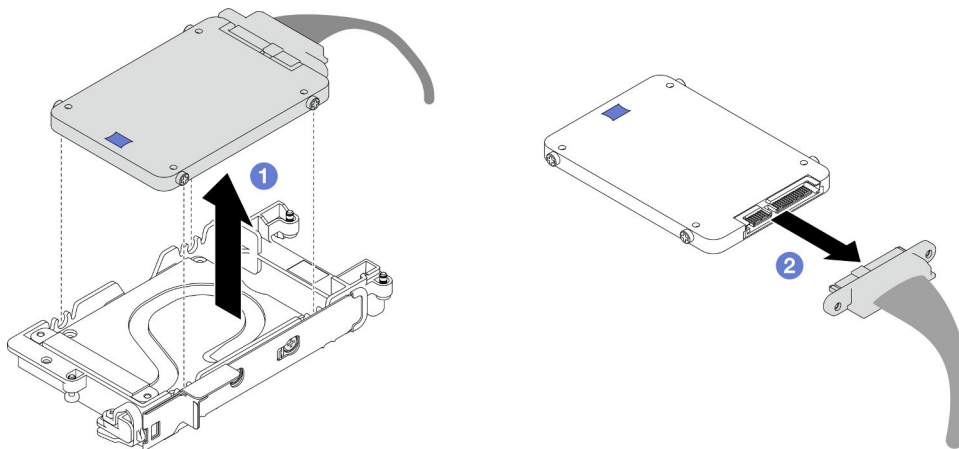
Figure 103. Retrait de l'unité inférieure
