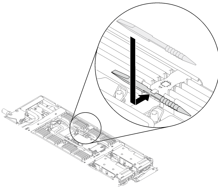
Figure 74. Installation de l'outil du module de mémoire
