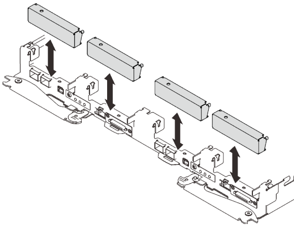
Figure 199. Retrait de l'obturateur vide du panneau
