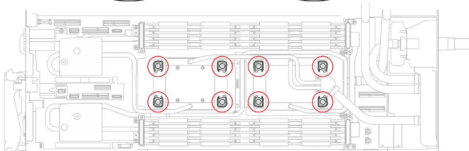
Figure 32. Desserrage des vis imperdables Torx T30
