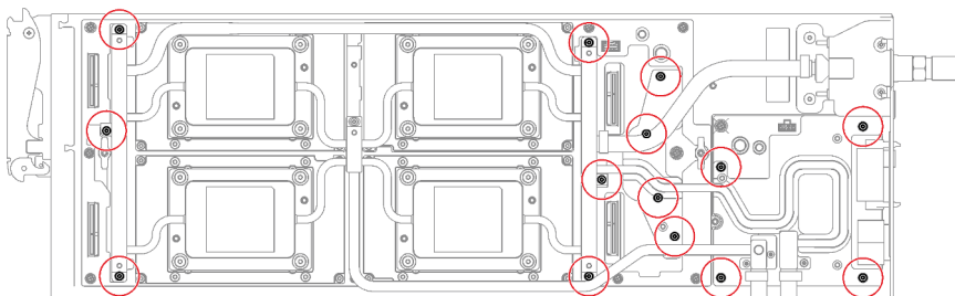
Figure 297. Retrait des vis de la boucle d'eau
