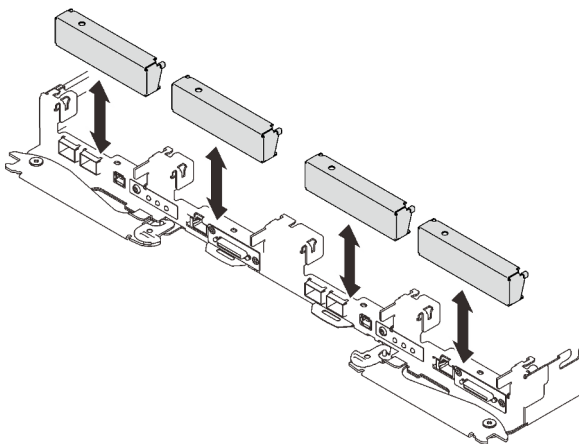
Figure 79. Installation de l'obturateur du panneau
