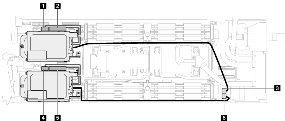
Figure 135. Cheminement des câbles de l'unité E3.S
