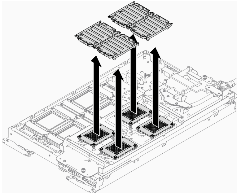
Figure 55. Retrait des films de protection en pâte thermoconductrice
