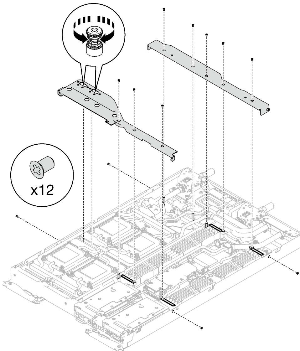
Figure 23. Retrait des traverses (SD650-I V3)
