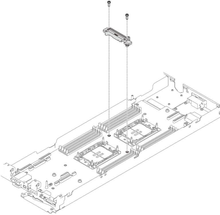
Figure 247. Retrait de la goulotte de la boucle d'eau VR
