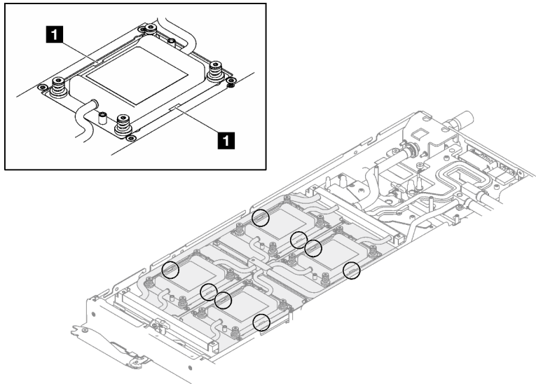
Figure 299. Encoches sur la plaque froide du GPU OAM
