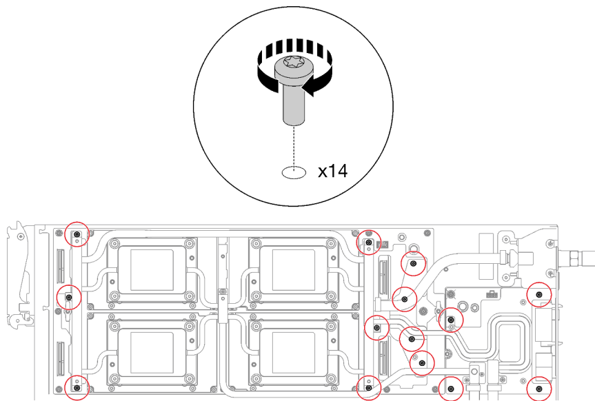
Figure 290. Installation des vis de la boucle d'eau
