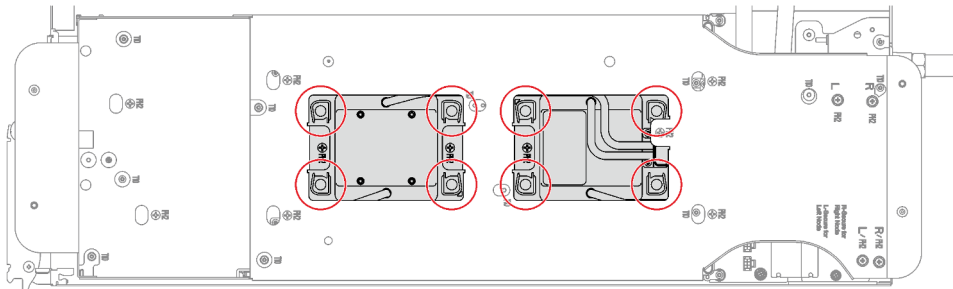
Figure 208. Desserrage des processeurs
