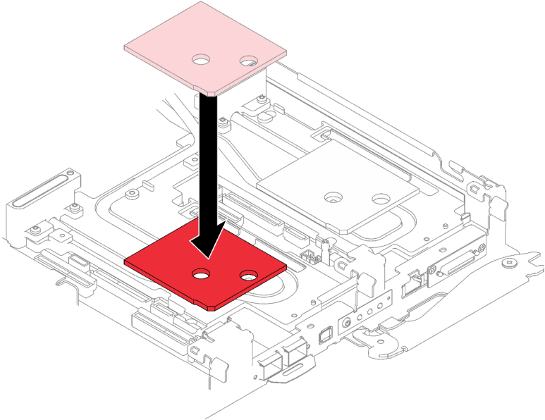
Figure 93. Remplacement du tampon d'espace
