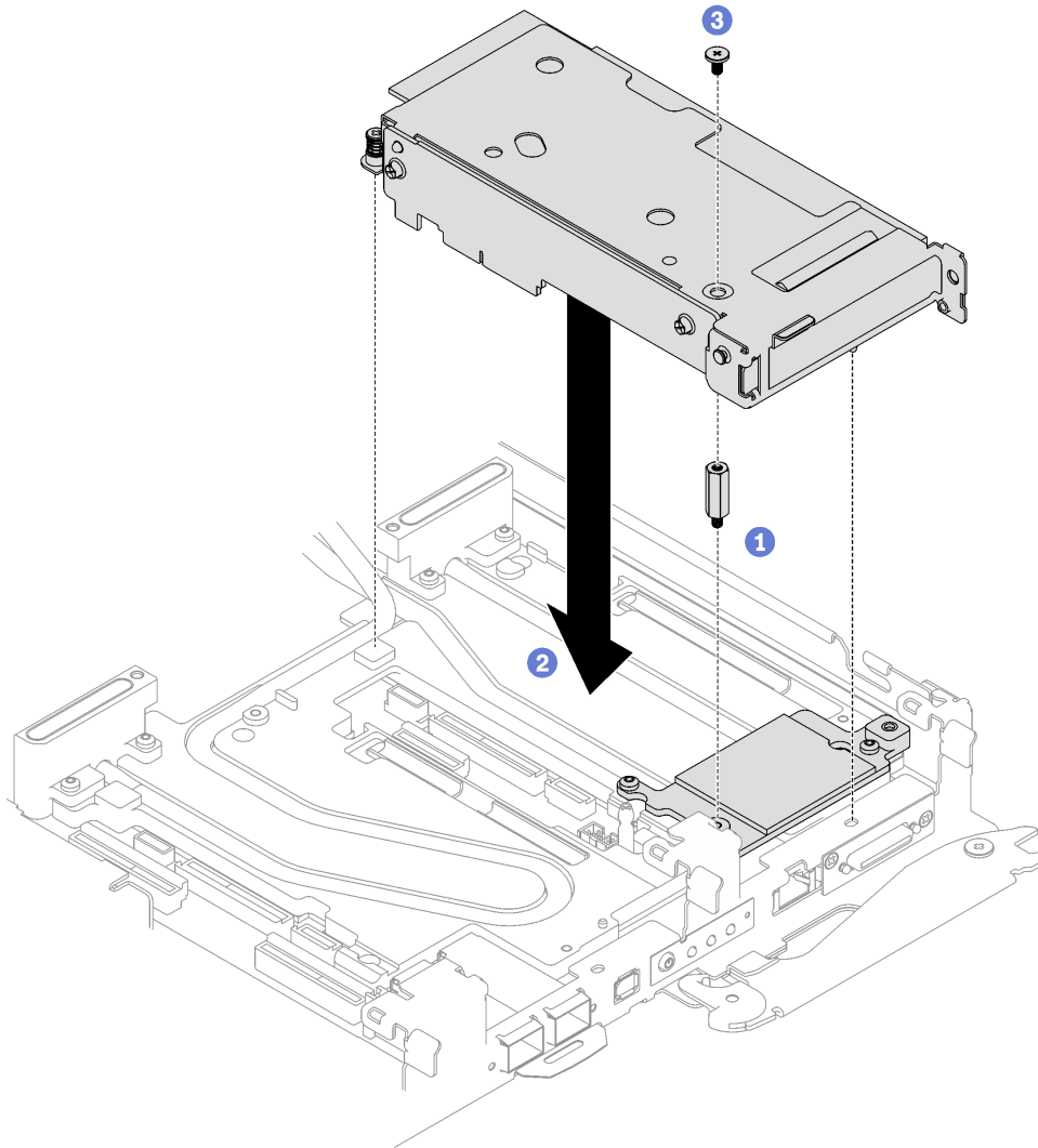
Figure 174. Installation de l'assemblage de cartes mezzanines PCIe
