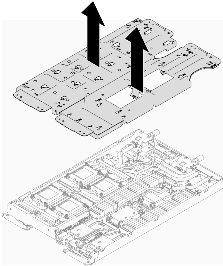
Figure 60. Retrait du support de la boucle d'eau
