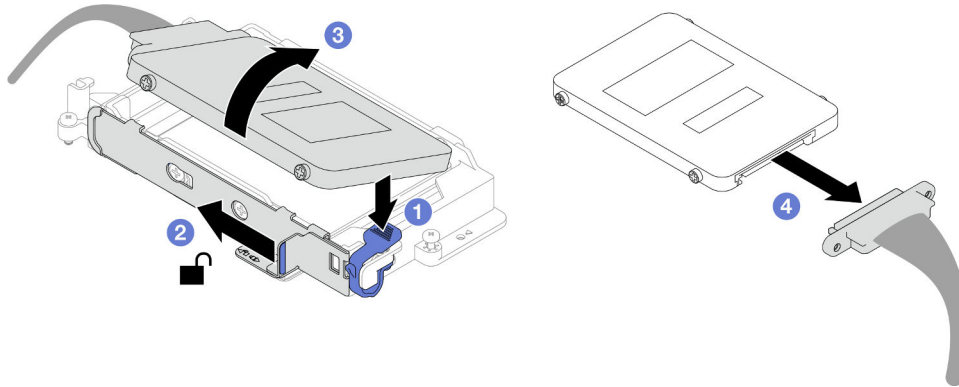
Figure 102. Retrait d'unité supérieure (NVMe 7 mm)
