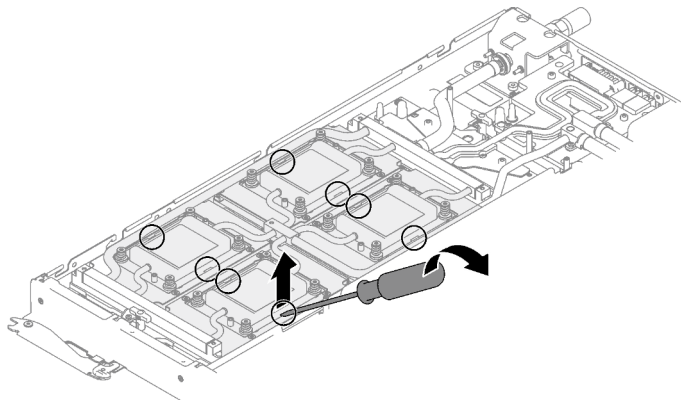
Figure 260. Libération de la plaque froide du GPU OAM
