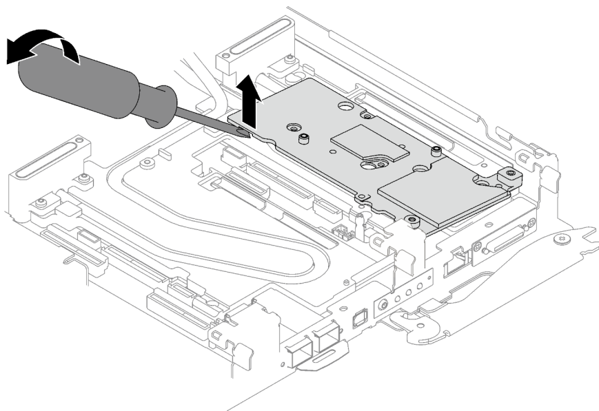
Figure 181. Libération de la plaque d'interface de la plaque froide de la boucle d'eau
