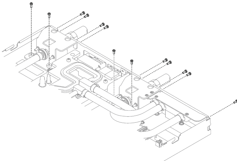
Figure 27. Retrait des vis du raccord rapide
