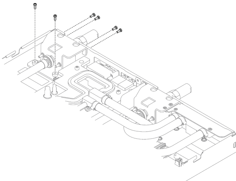
Figure 296. Retrait des vis du raccord rapide
