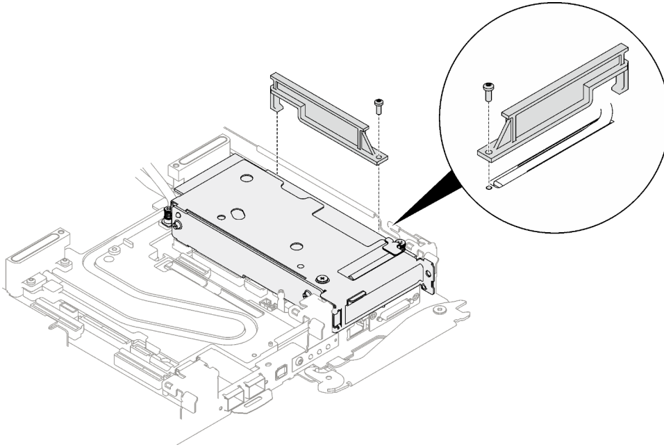
Figure 165. Retrait du profilé du tube thermique
