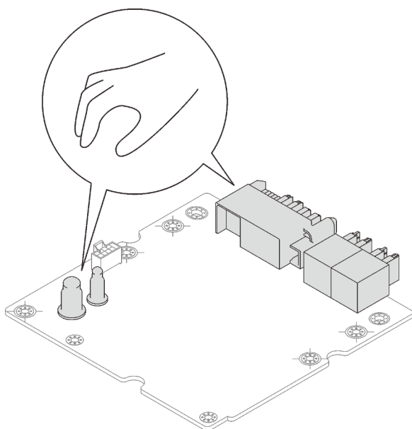
Figure 306. Points de contact du tableau de distribution du GPU SD650-I V3
