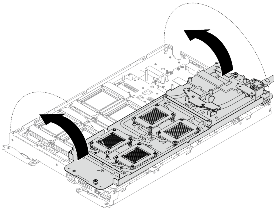
Figure 287. Installation de la boucle d'eau
