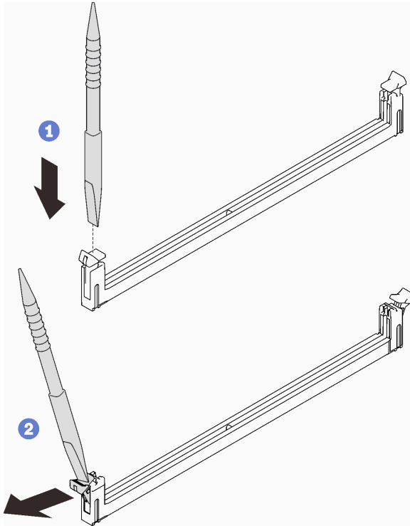
Figure 156. Pression sur les clips de retenue sur le connecteur du module de mémoire
