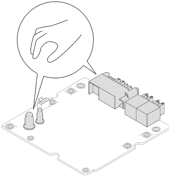
Figure 295. Points de contact du tableau de distribution du GPU SD650-I V3
