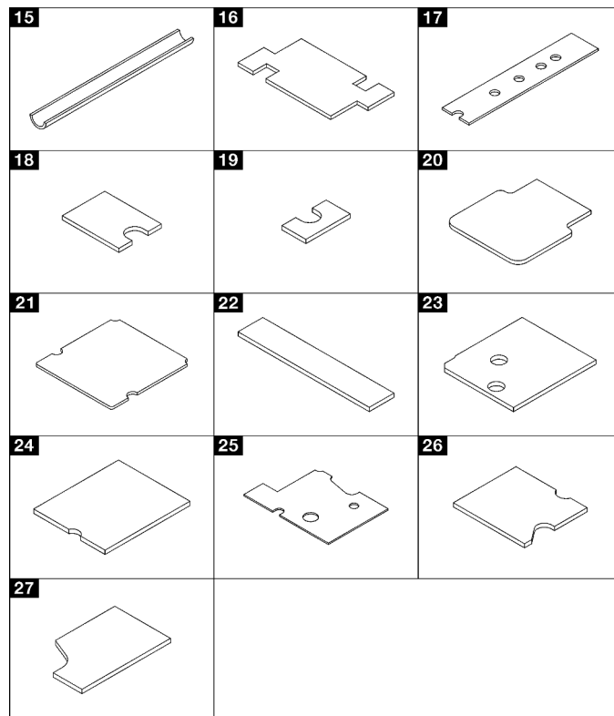
Figure 17. Tampons d'espace et tampons de mastic utilisés dans le SD650-I V3
