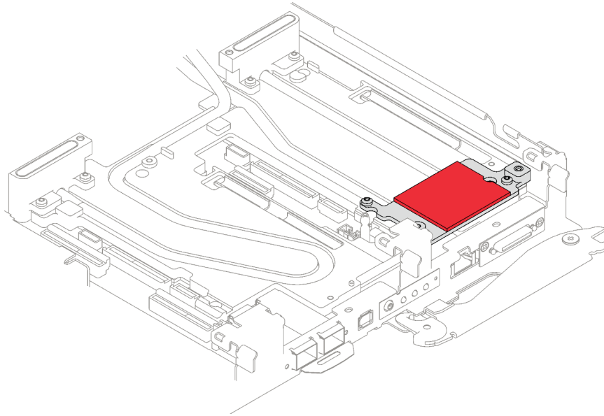
Figure 173. Tampon de mastic de la plaque d'interface pour carte mezzanine CX-6
