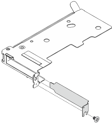
Figure 161. Installation de l'obturateur
