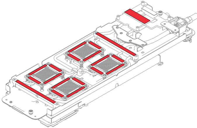
Figure 269. Emplacements des tampons de mastic
