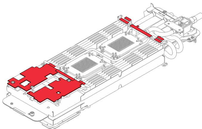
Figure 49. Tampons d'espace de la boucle d'eau
