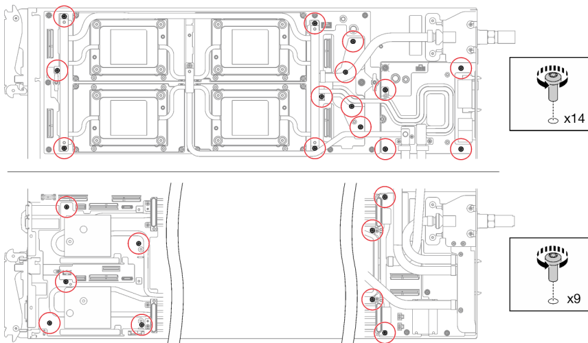
Figure 28. Retrait des vis de la boucle d'eau
