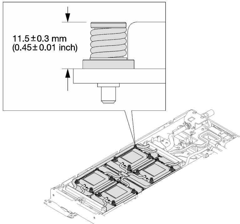
Figure 319. Hauteur de la vis de la plaque froide du GPU OAM correctement installée
