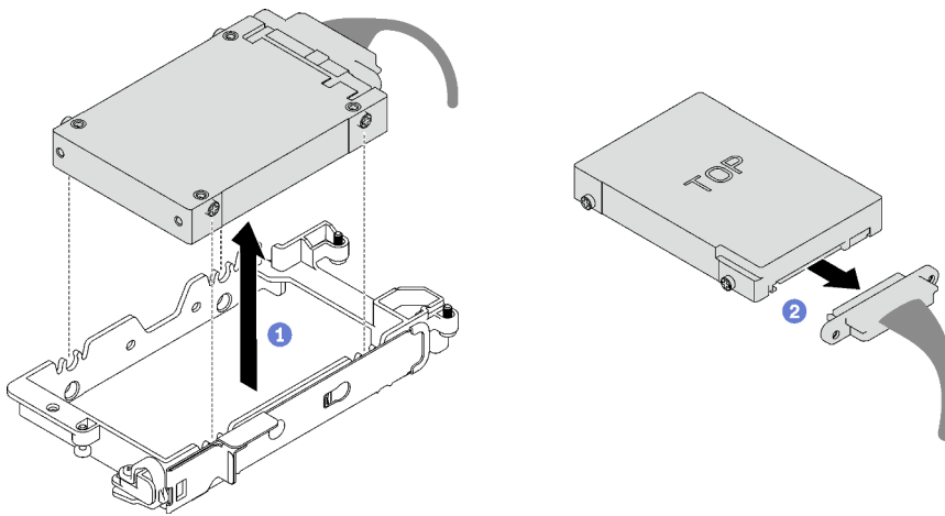
Figure 81. Retrait d'une unité 15 mm
