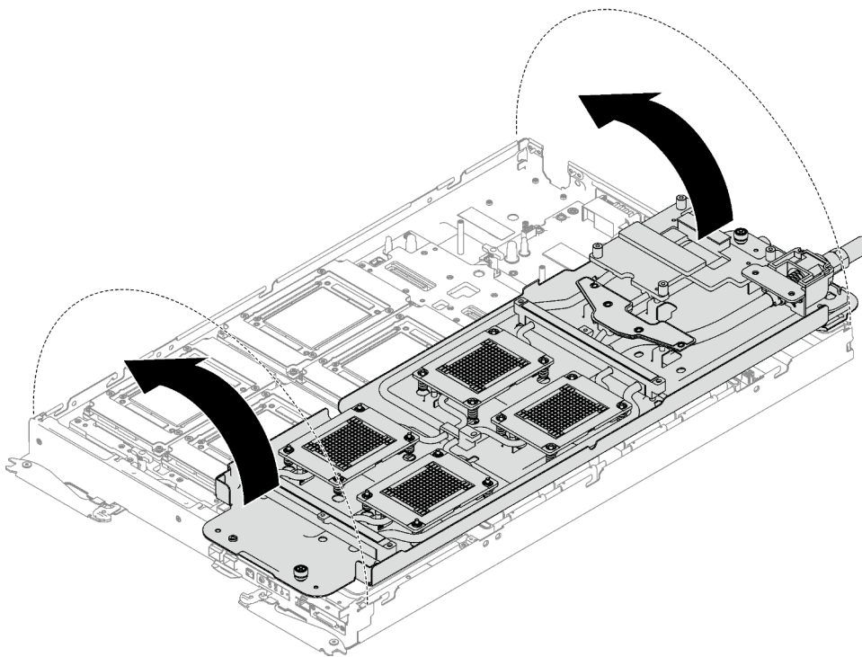
Figure 312. Installation de la boucle d'eau
