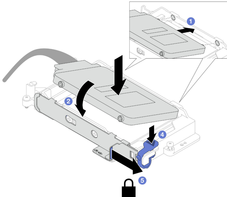
Figure 107. Installation de l'unité supérieure
