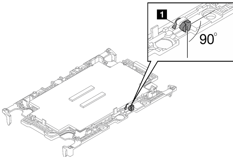
Figure 235. Came de rupture TIM sur le dispositif de retenue du processeur
