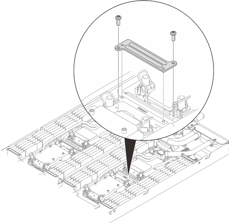
Figure 221. Retrait de la plaque de serrage VR
