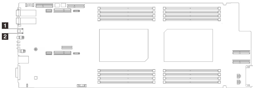
Figure 331. Voyants de la carte mère
