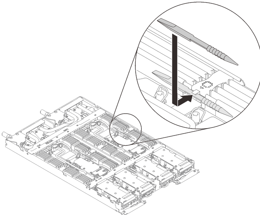
Figure 153. Installation de l'outil du module de mémoire
