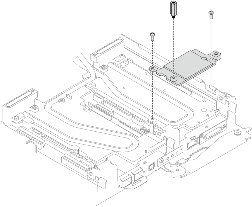
Figure 168. Retrait de la plaque d'interface
