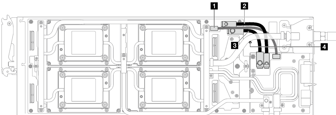
Figure 321. Cheminement des câbles du plateau SD650-I V3
