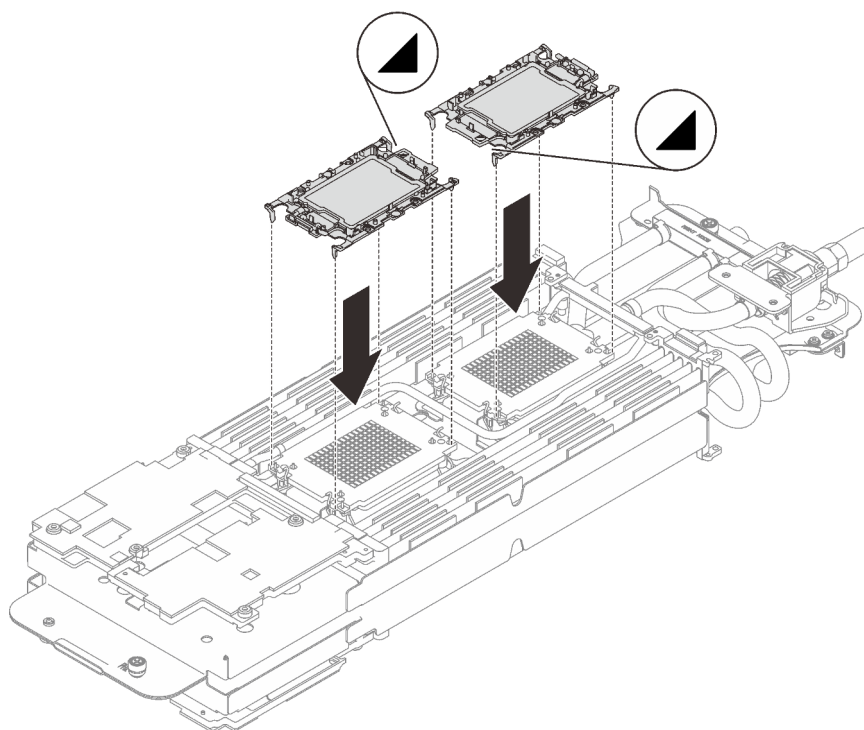
Figure 47. Installation d'un processeur
