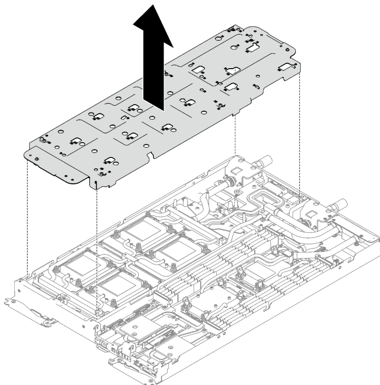
Figure 272. Retrait du support de la boucle d'eau
