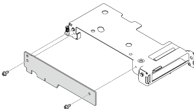
Figure 170. Retrait de la carte d'extension
