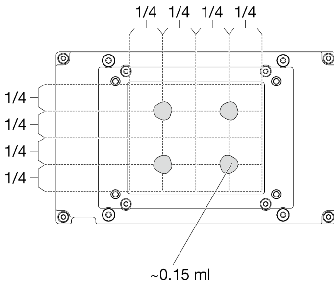
Figure 267. Application de la pâte thermoconductrice
