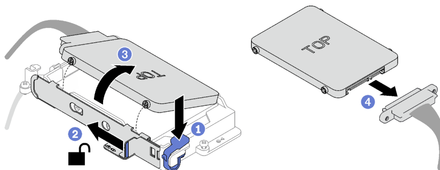
Figure 82. Retrait de l'unité supérieure
