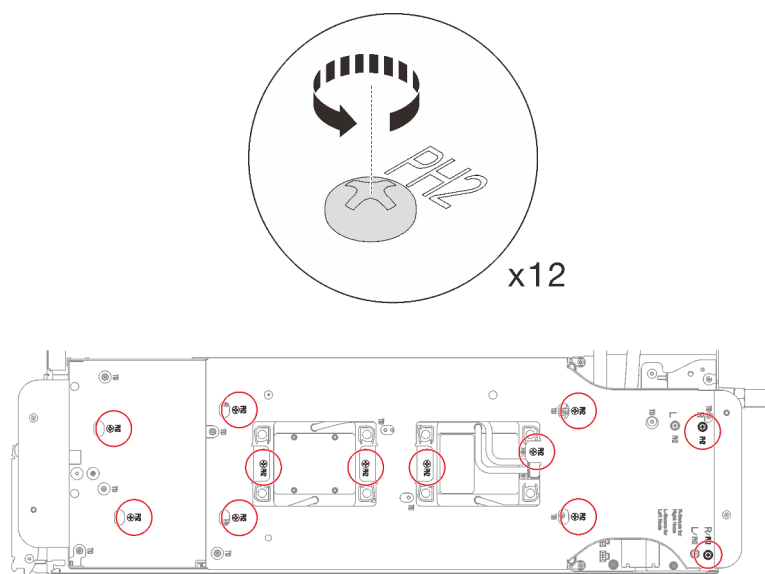
Figure 242. Desserrage des vis du support de la boucle d'eau
