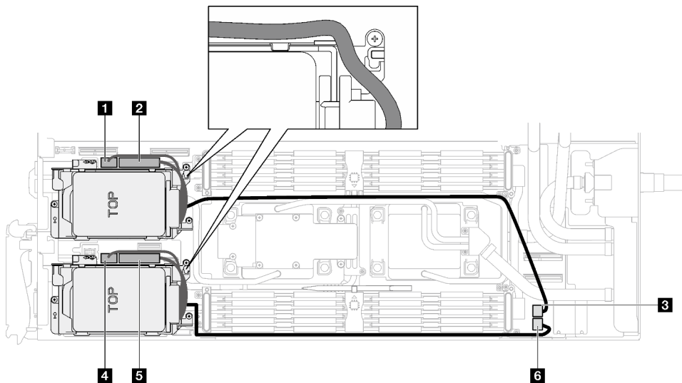
Figure 75. Cheminement des câbles du bloc unité
