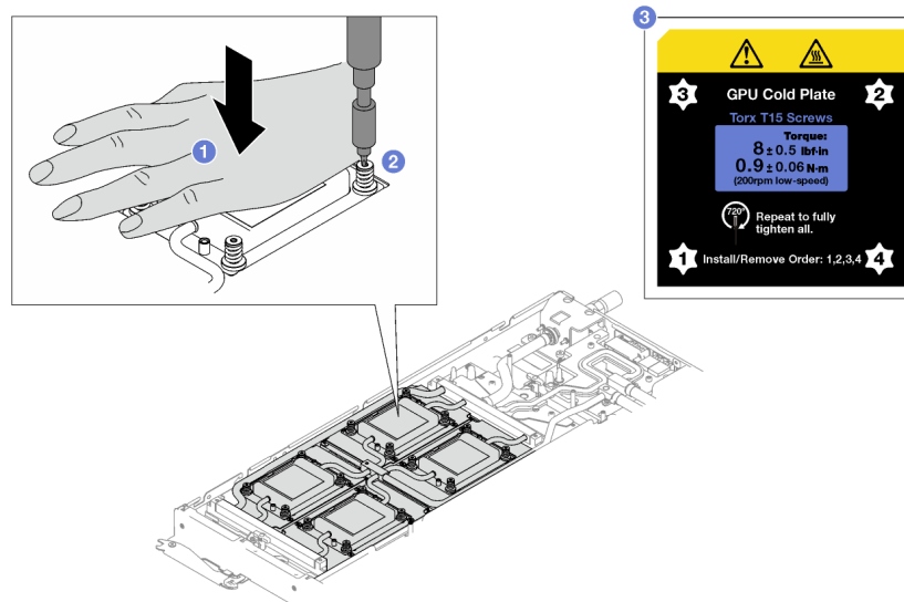
Figure 276. Serrage des vis de la plaque froide du GPU OAM sur 720 degrés
