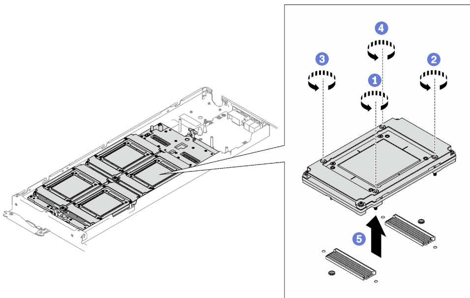
Figure 264. Retrait du GPU OAM
