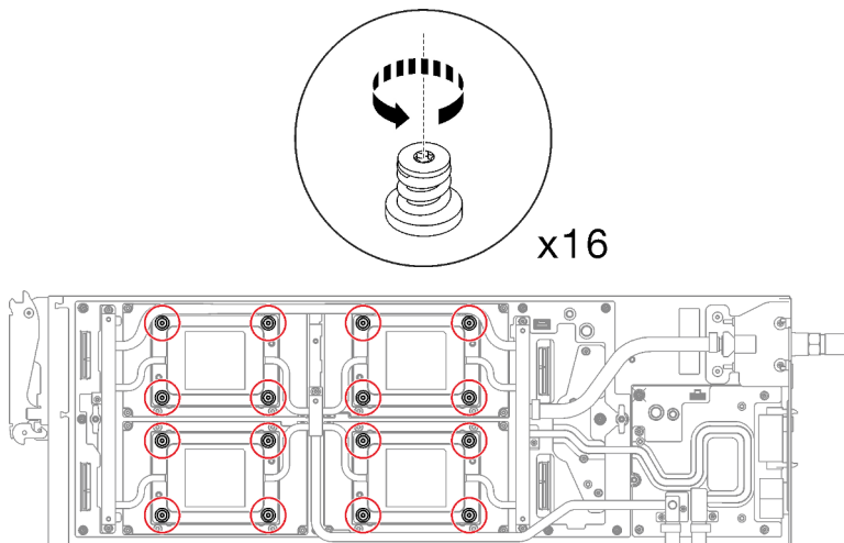
Figure 298. Retrait des vis de la plaque froide du GPU OAM
