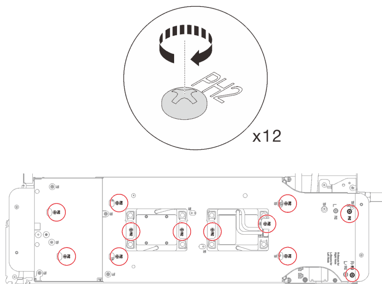
Figure 207. Installation des vis du support de boucle d'eau
