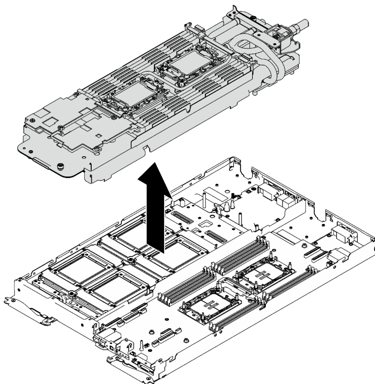
Figure 40. Retrait de la boucle d'eau
