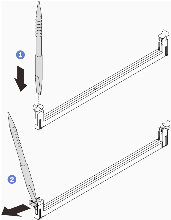
Figure 151. Pression sur les clips de retenue sur le connecteur du module de mémoire
