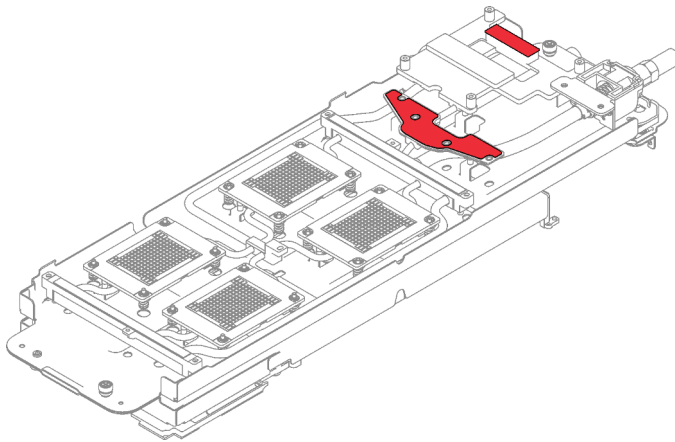
Figure 310. Tampons d'espace de la boucle d'eau
