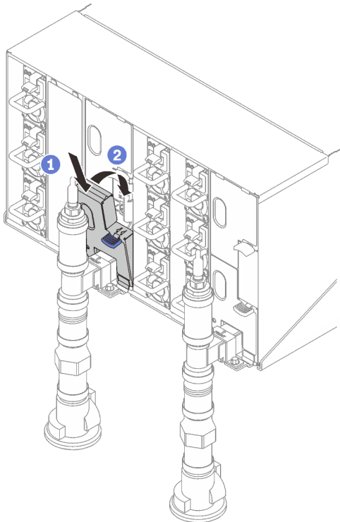
Figure 336. Installation d'un blindage électromagnétique
