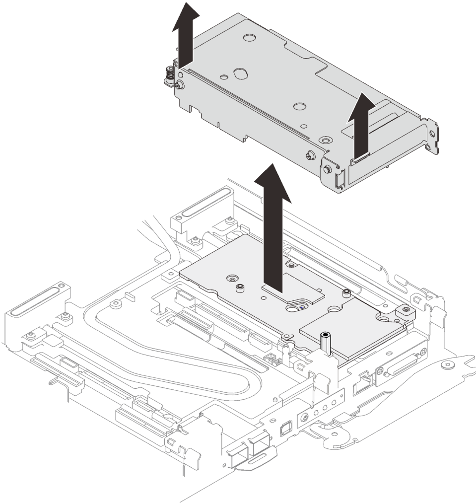
Figure 178. Retrait de l'assemblage de cartes mezzanines PCIe
