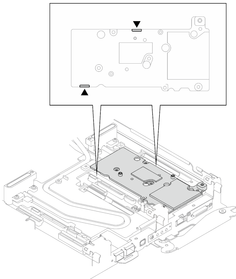
Figure 180. Emplacements des ouvertures sur la partie inférieure de la plaque d'interface
