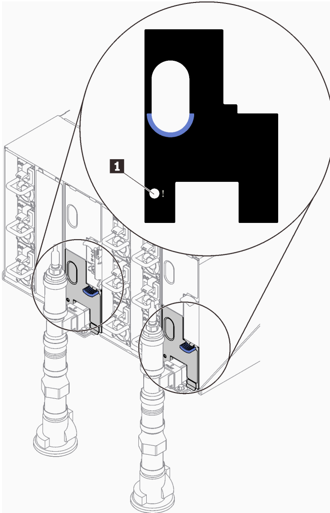
Figure 332. Voyant du capteur de gouttes
