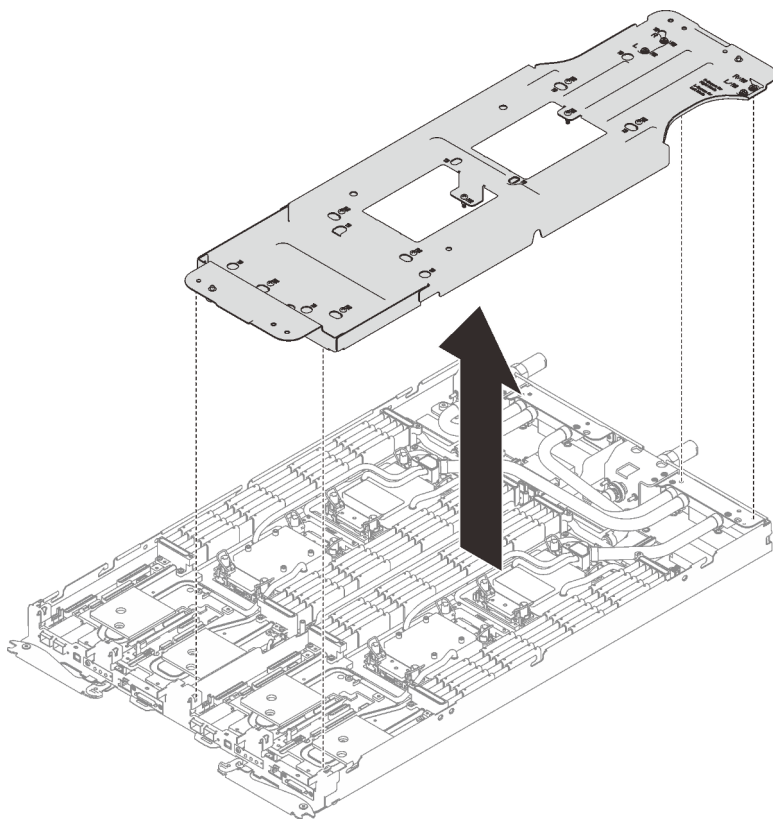
Figure 243. Retrait du support de la boucle d'eau
