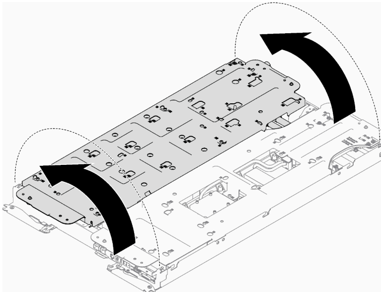
Figure 57. Dépliage de la boucle d'eau
