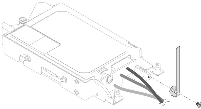
Figure 118. Retrait de l'attache-câbles
