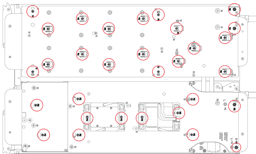
Figure 34. Installation des vis du support de boucle d'eau
