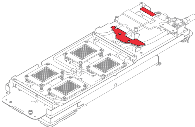
Figure 268. Tampons d'espace de la boucle d'eau
