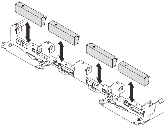
Figure 169. Installation de l'obturateur du panneau
