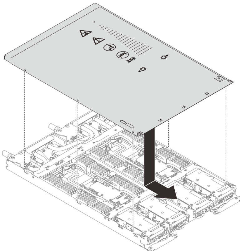
Figure 21. Installation du cache du plateau
