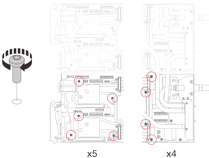
Figure 244. Installation des vis de la boucle d'eau
