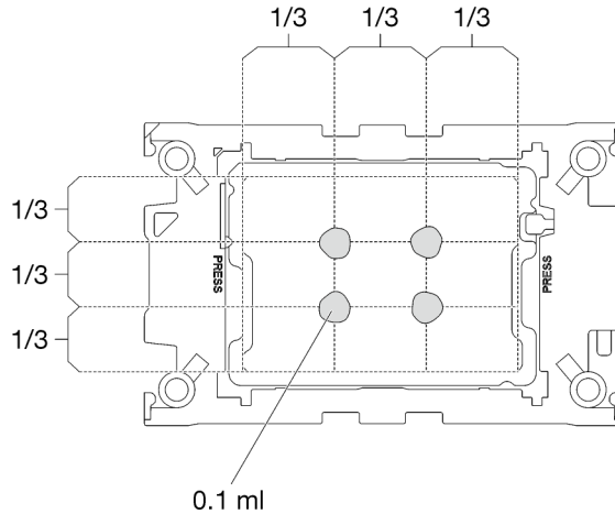
Figure 41. Application de la pâte thermoconductrice
