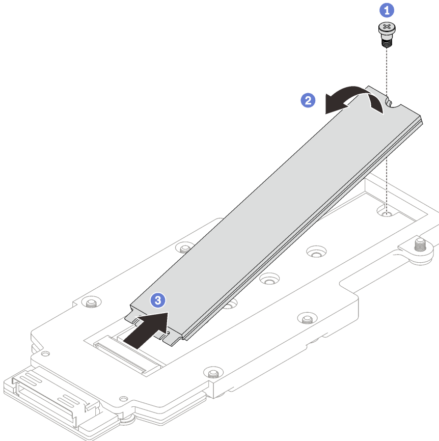
Figure 142. Retrait d'une unité M.2
