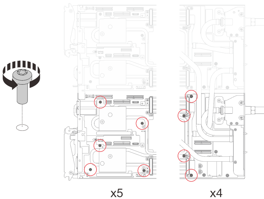
Figure 204. Retrait des vis de la boucle d'eau
