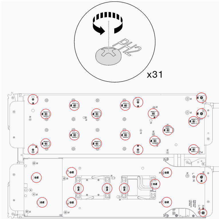
Figure 59. Desserrage des vis du support de la boucle d'eau
