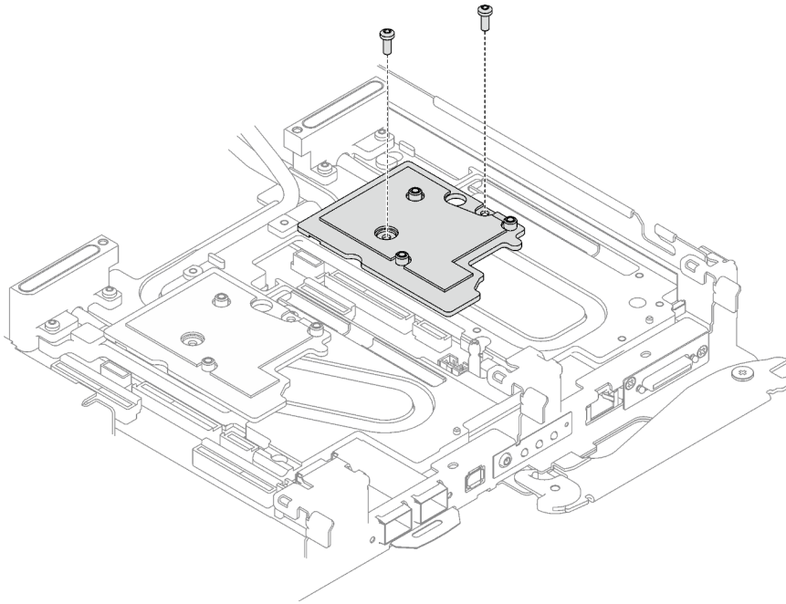
Figure 200. Installation de la plaque d'interface
