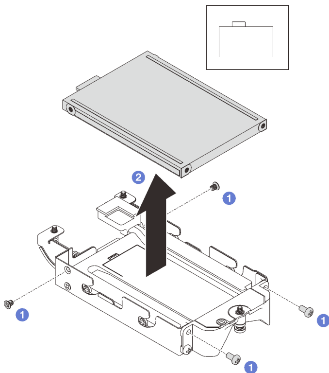
Figure 120. Retrait de l'unité E3.S inférieure
