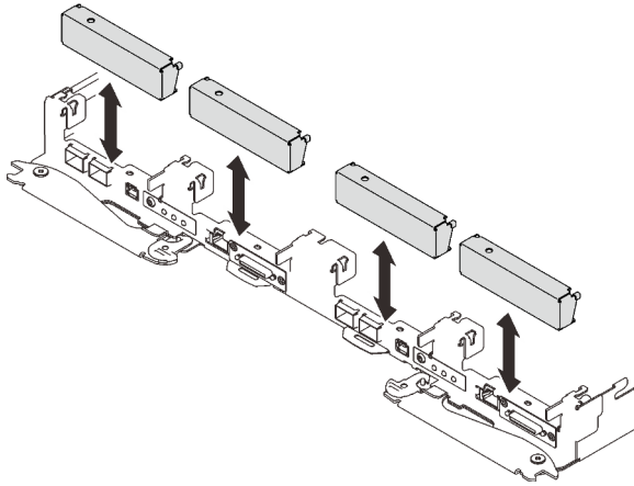
Figure 197. Installation de l'obturateur du panneau
