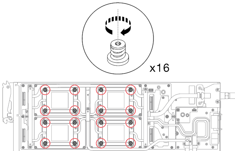
Figure 275. Installation des vis de la plaque froide du GPU OAM
