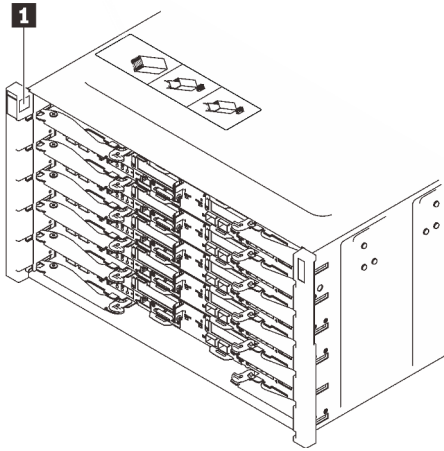
Figure 12. Étiquette du boîtier à l'avant du boîtier
