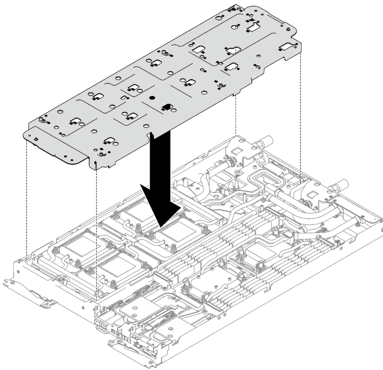
Figure 261. Installation du support de boucle d'eau
