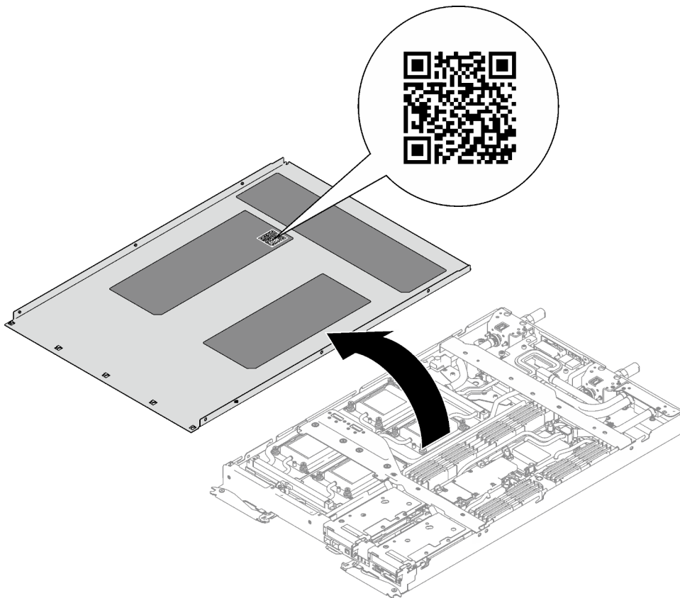
Figure 15. Étiquette de maintenance et code QR
