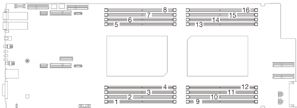
Figure 149. Emplacement du connecteur du module de mémoire
