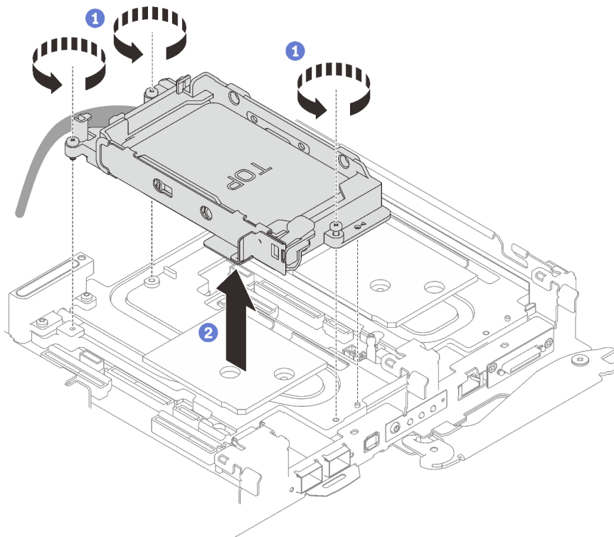
Figure 77. Retrait d'un bloc boîtier d'unités de disque dur 7 mm
