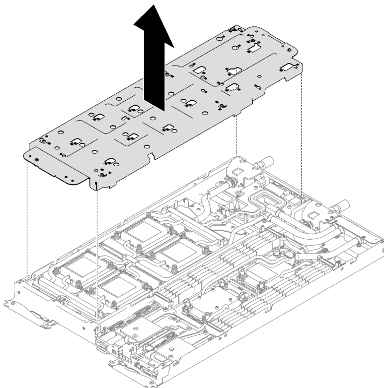
Figure 289. Retrait du support de la boucle d'eau
