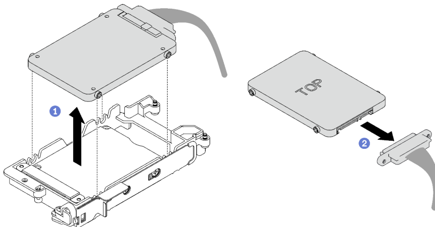
Figure 80. Retrait d'une unité 7 mm
