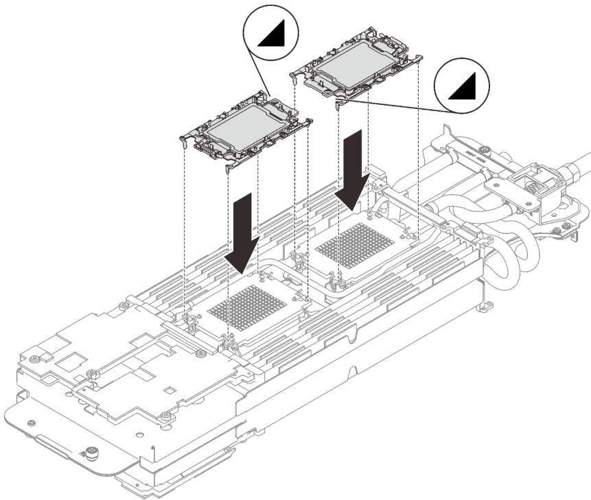
Figure 237. Installation d'un processeur
