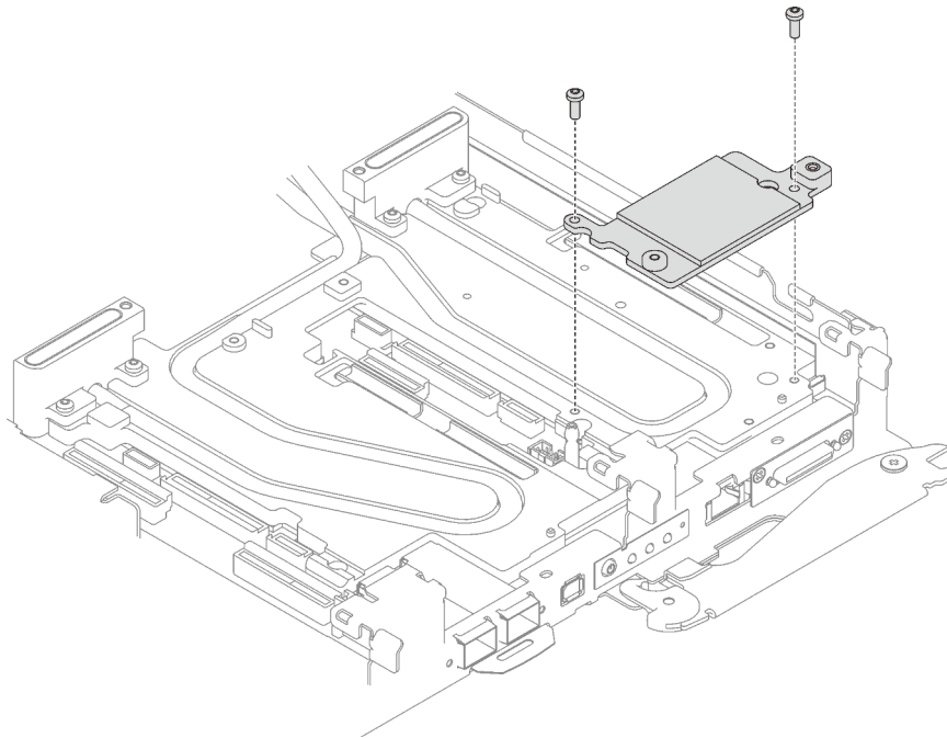
Figure 172. Installation de la plaque d'interface
