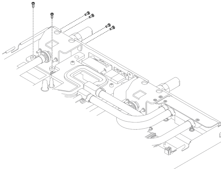
Figure 274. Installation des vis du raccord rapide
