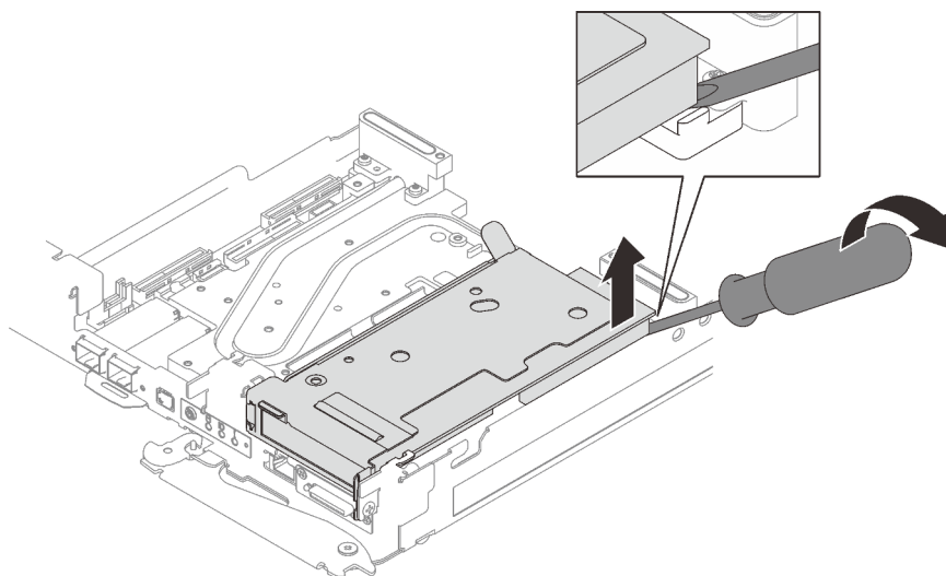
Figure 191. Libération de la cage de carte mezzanine PCIe de la plaque froide de la boucle d'eau
