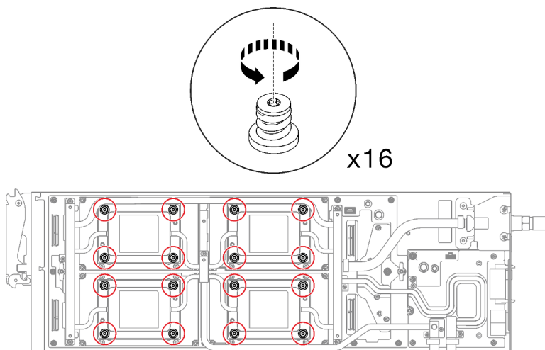
Figure 29. Retrait des vis de la plaque froide du GPU OAM
