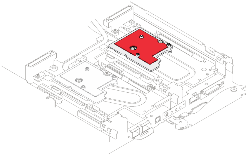
Figure 201. Tampon d'espace sur la plaque d'interface pour CX-7 NDR 400
