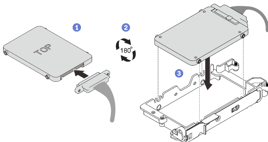
Figure 88. Installation de l'unité inférieure
