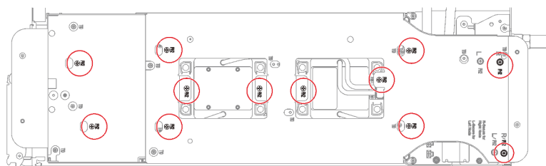
Figure 225. Installation des vis du support de boucle d'eau
