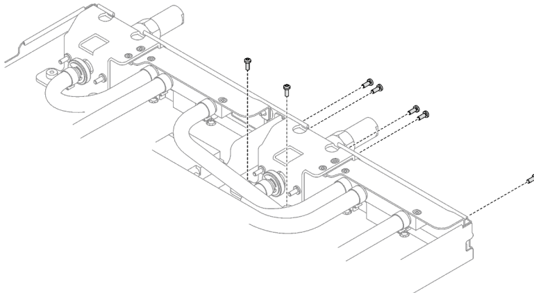
Figure 223. Retrait des vis du raccord rapide
