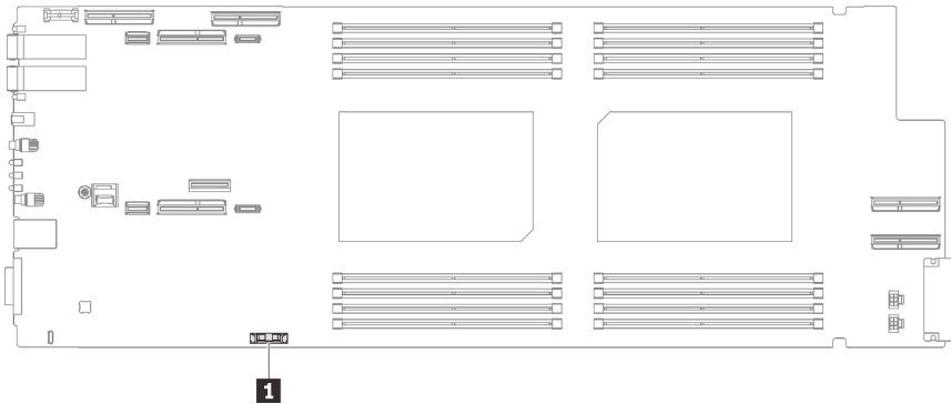
Figure 69. Emplacement de la pile CMOS
