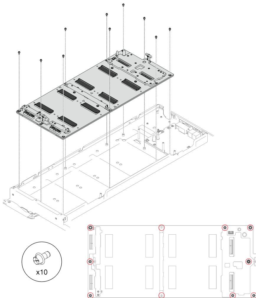
Figure 278. Retrait des vis
