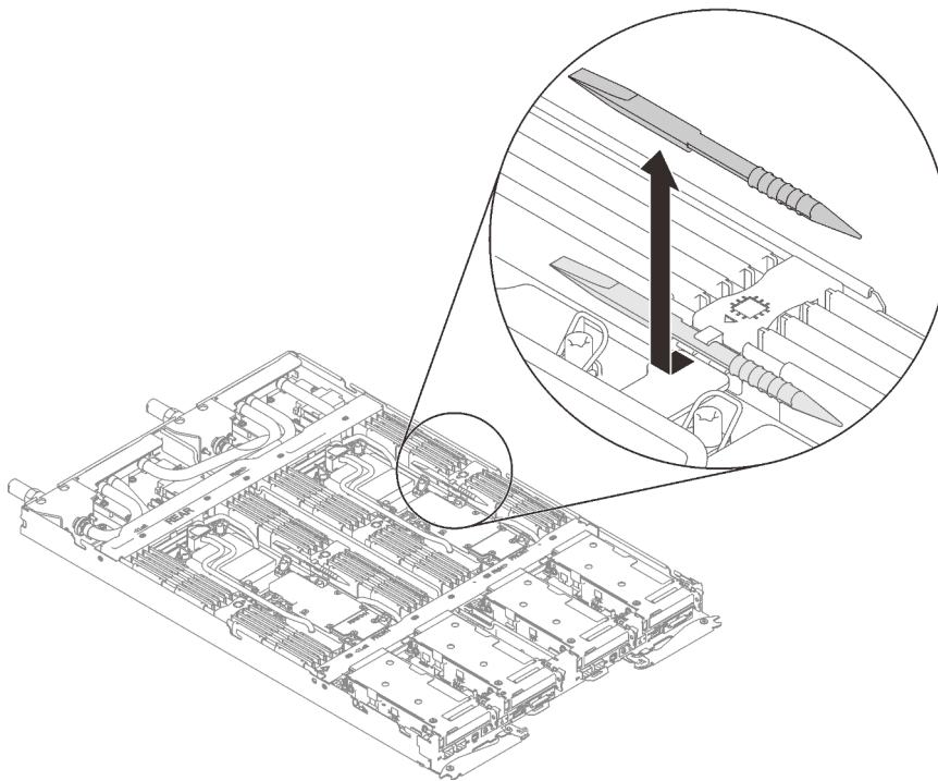
Figure 150. Retrait de l'outil du module de mémoire
