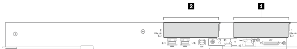
Figure 9. Numérotation des emplacements PCIe - Plateau SD650-I V3
