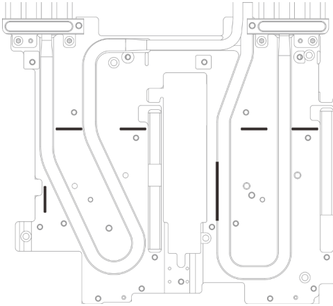
Figure 92. Marquages sur la boucle d'eau pour aligner le tampon d'espace
