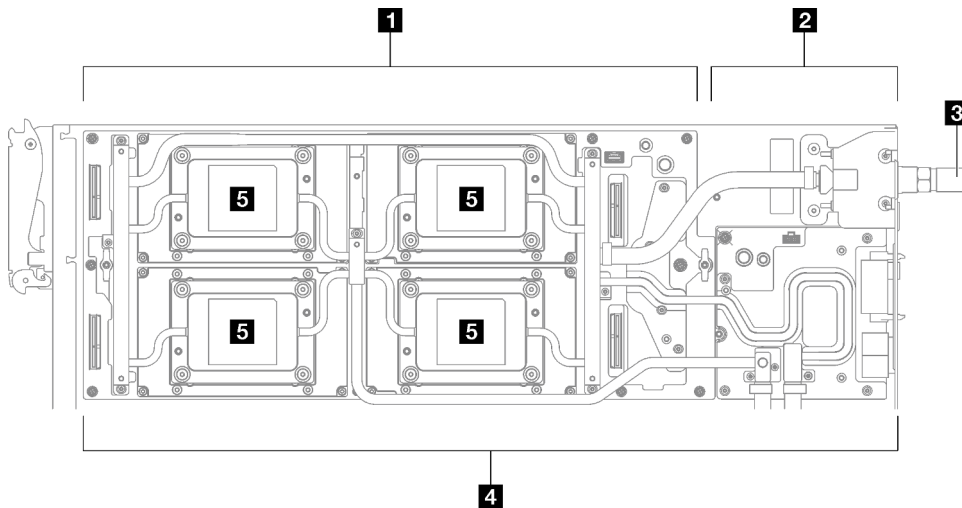
Figure 4. Vue supérieure du nœud GPU
