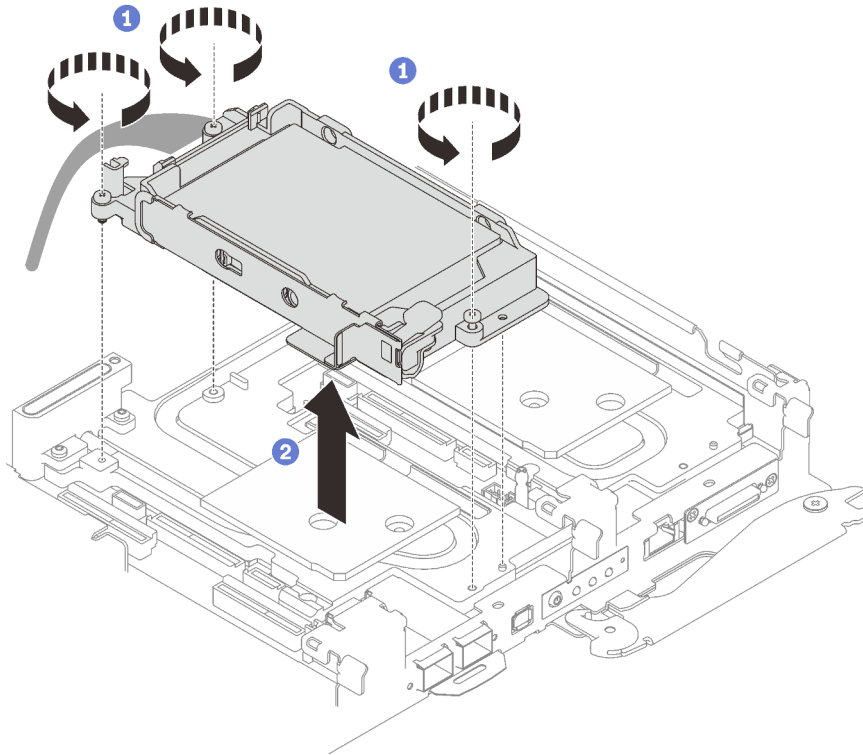
Figure 76. Retrait d'un bloc boîtier d'unités de disque dur 15 mm
