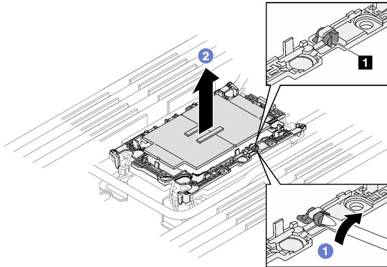
Figure 229. Retrait d'un processeur (processeur Intel® Xeon® CPU Max)
