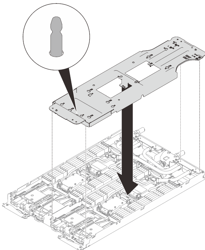
Figure 224. Installation du support de boucle d'eau
