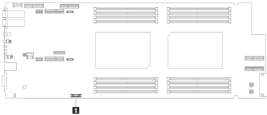
Figure 67. Emplacement de la pile CMOS
