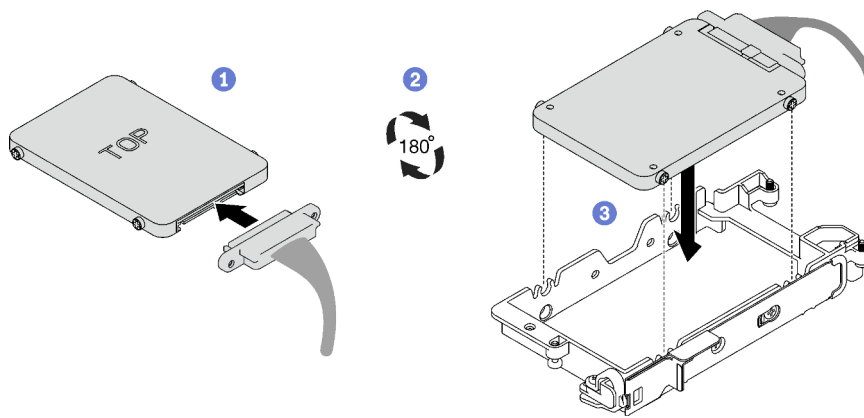
Figure 85. Installation de l'unité 7 mm
