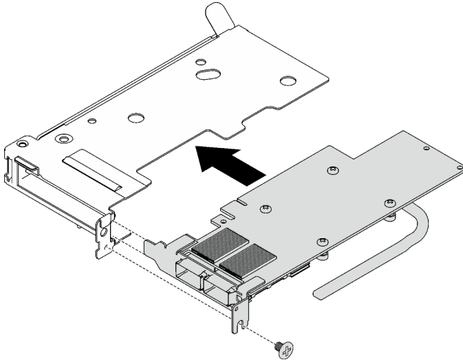
Figure 164. Installer un adaptateur PCIe
