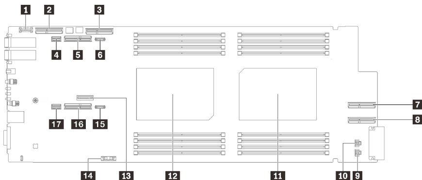
Figure 6. Connecteurs internes de la carte mère du nœud de traitement
