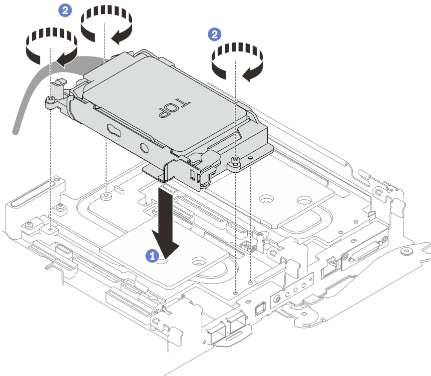
Figure 97. Installation de deux blocs boîtier d'unités de disque dur 7 mm
