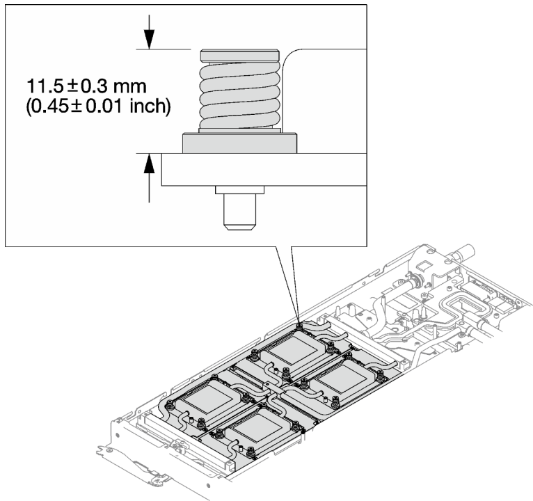
Figure 65. Hauteur de la vis de la plaque froide du GPU OAM correctement installée
