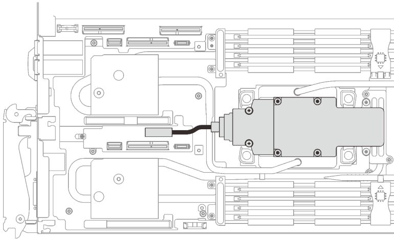
Figure 138. Retrait du câble du fond de panier M.2
