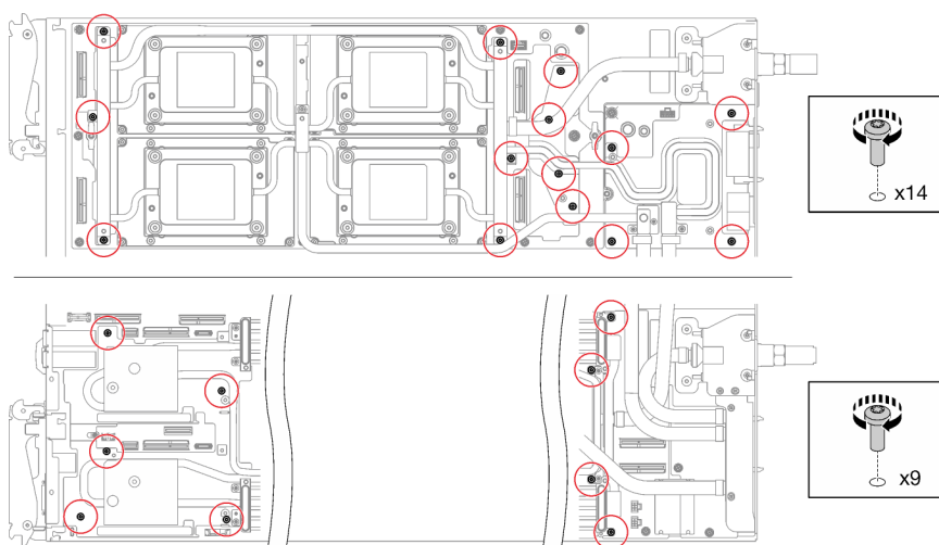
Figure 61. Installation des vis de la boucle d'eau
