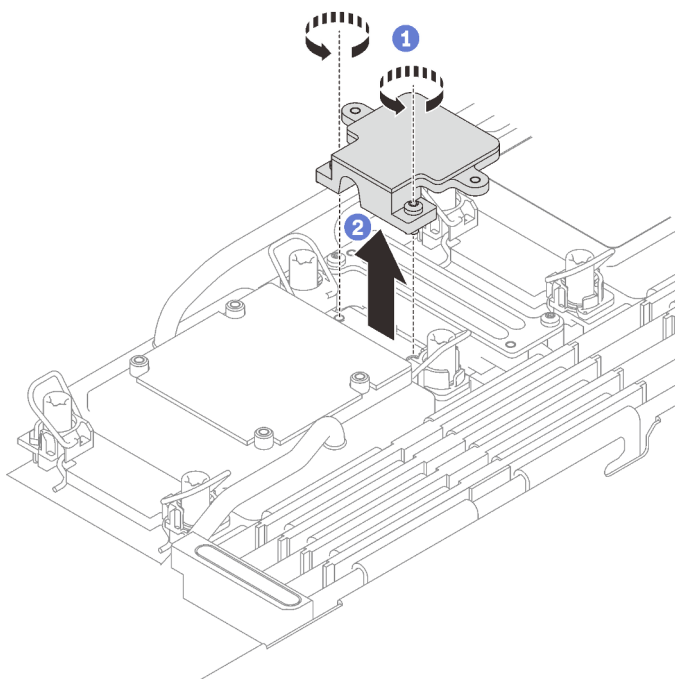
Figure 140. Retrait de la plaque froide du fond de panier M.2
