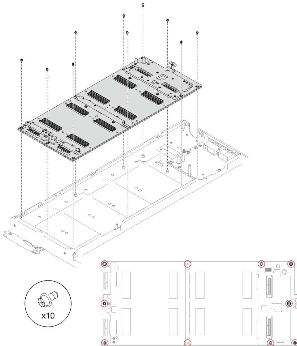
Figure 282. Installation de la carte de base du support
