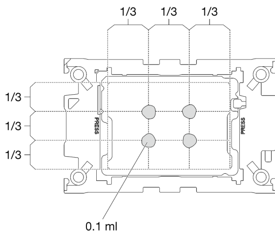
Figure 232. Application de la pâte thermoconductrice
