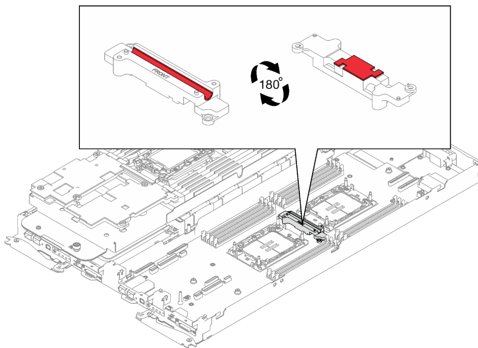
Figure 253. Tampons d'espace de la goulotte de la boucle d'eau VR
