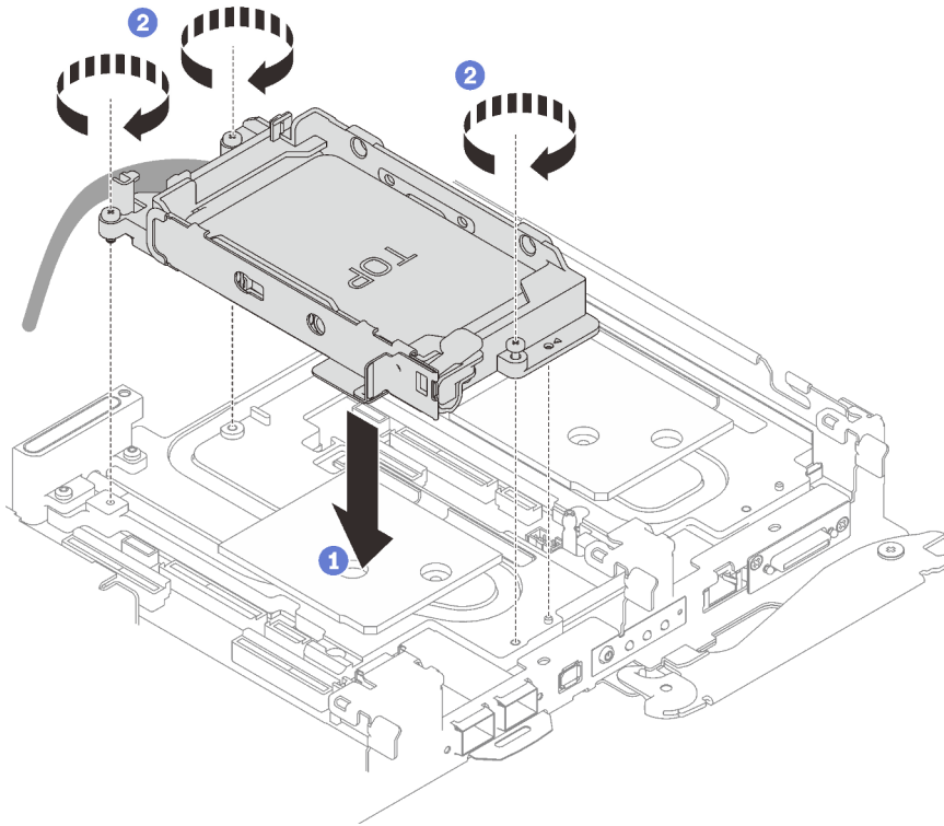
Figure 96. Installation d'un bloc boîtier d'unités de disque dur 7 mm
