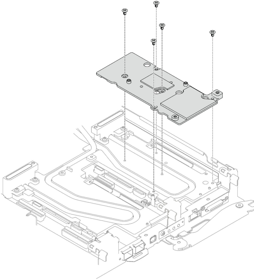
Figure 186. Installation de la plaque d'interface
