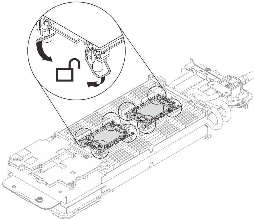
Figure 238. Position déverrouillée du processeur
