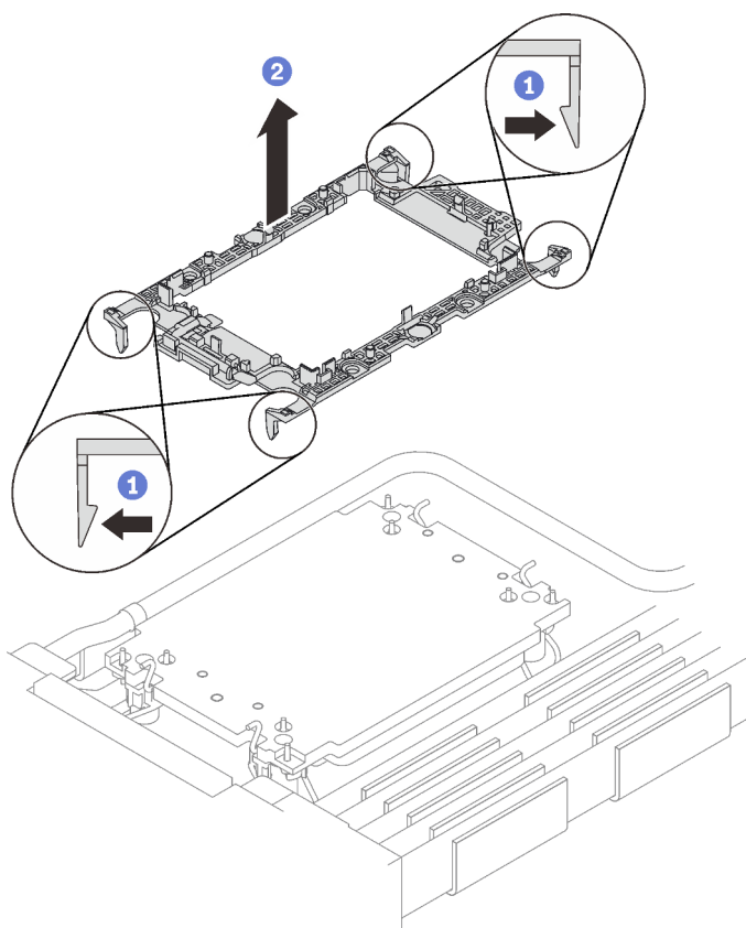
Figure 39. Retrait du dispositif de retenue du processeur
