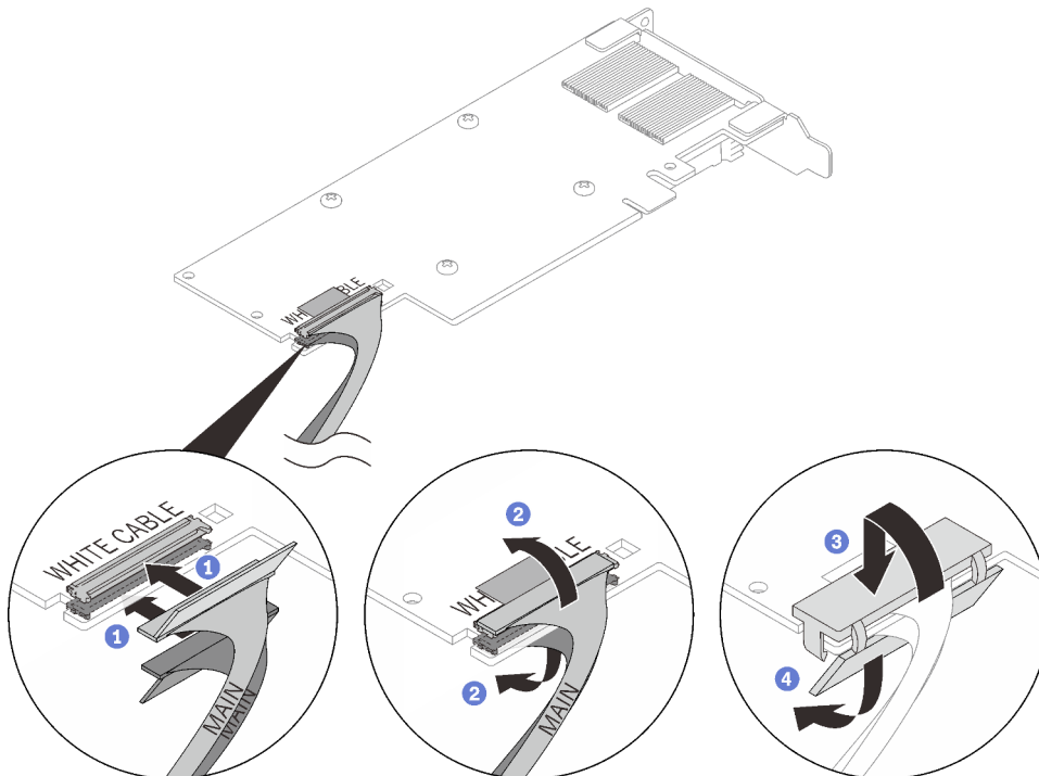
Figure 163. Installation des câbles d'adaptateur PCIe
