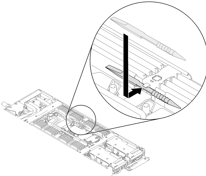
Figure 158. Installation de l'outil du module de mémoire
