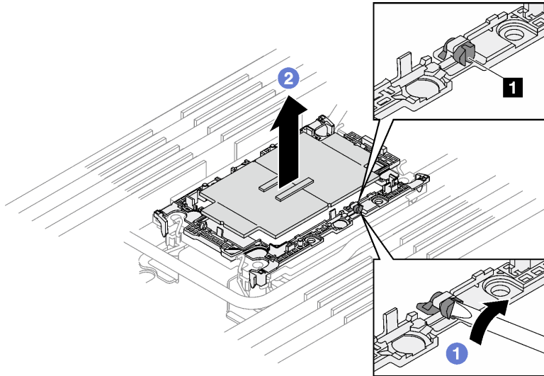
Figure 38. Retrait d'un processeur (processeur Intel® Xeon® CPU Max)
