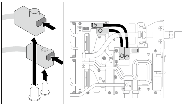
Figure 320. Connecteur du cordon d'alimentation
