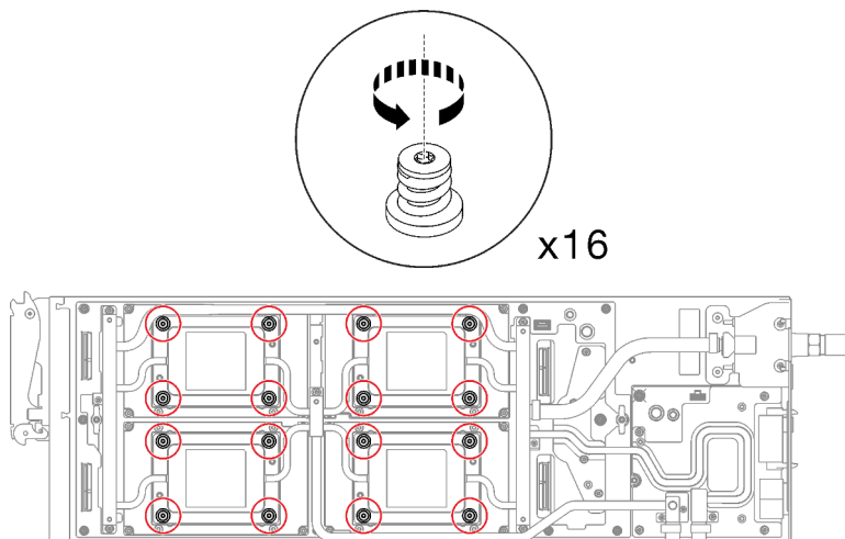
Figure 258. Retrait des vis de la plaque froide du GPU OAM
