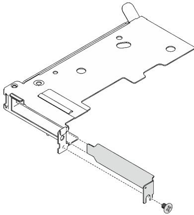
Figure 162. Retrait de l'obturateur
