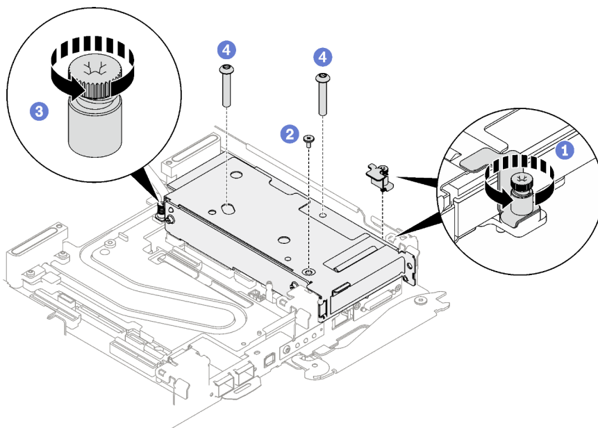
Figure 177. Retrait de la vis imperdable de l'étrier de fixation
