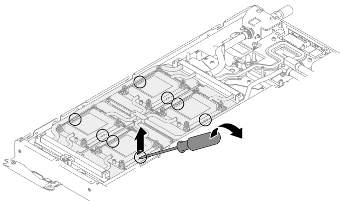
Figure 31. Libération de la plaque froide du GPU OAM
