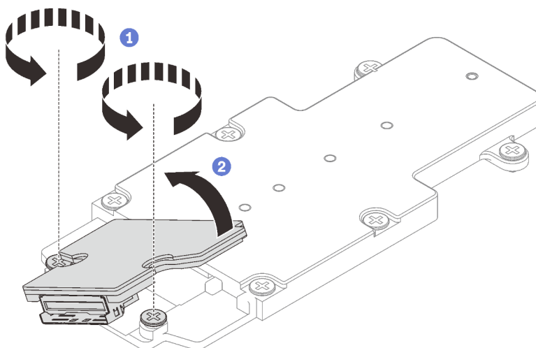
Figure 141. Démontage du fond de panier M.2
