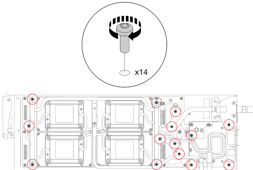
Figure 273. Installation des vis de la boucle d'eau
