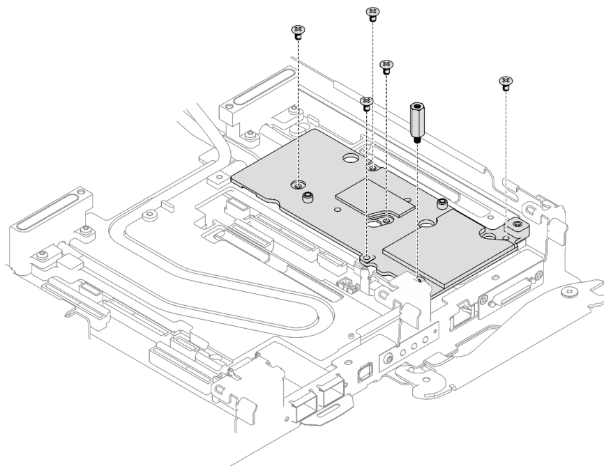
Figure 179. Retrait de la plaque d'interface
