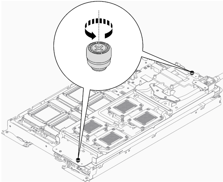
Figure 56. Desserrement des vis moletées imperdables
