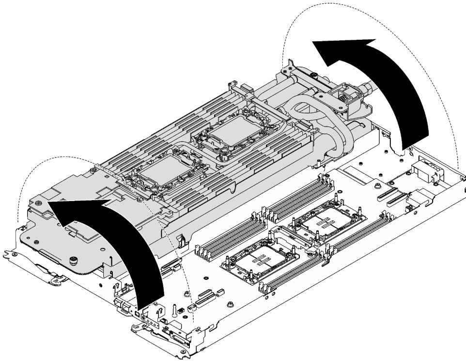
Figure 35. Plier la boucle d'eau
