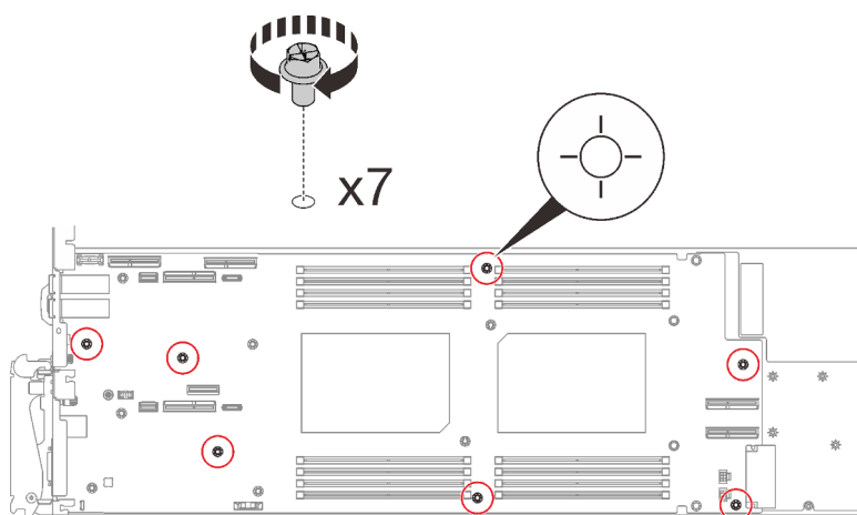
Figure 252. Installation des vis de la carte mère
