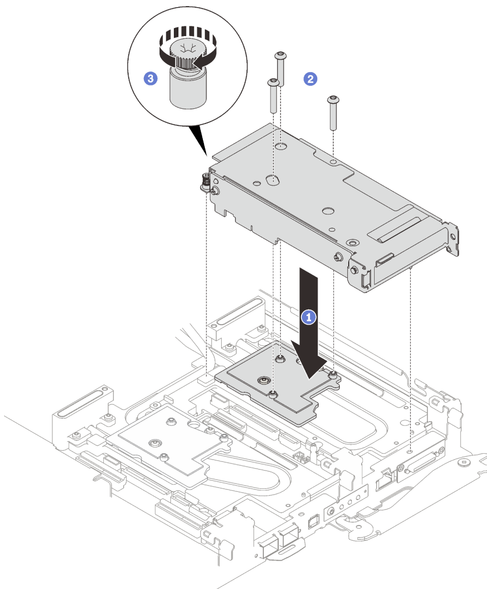
Figure 202. Installation de l'assemblage de cartes mezzanines PCIe
