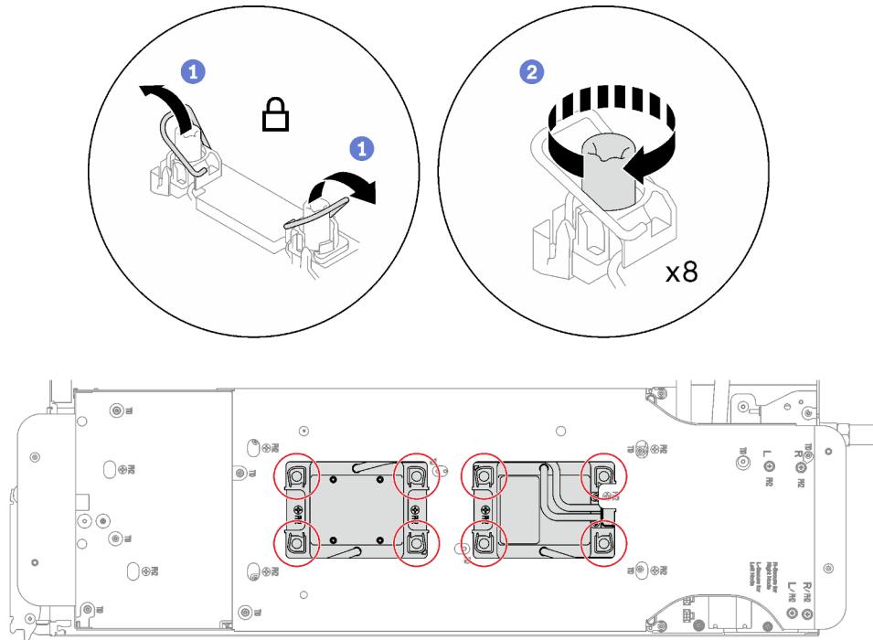
Figure 214. Installation des processeurs
