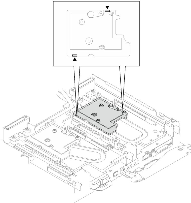
Figure 194. Emplacements des ouvertures sur la partie inférieure de la plaque d'interface
