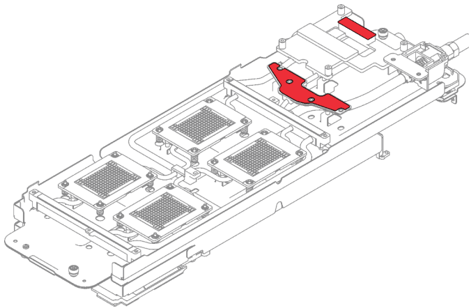
Figure 285. Tampons d'espace de la boucle d'eau
