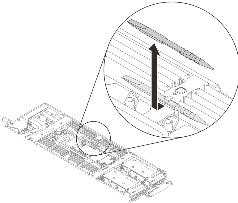
Figure 155. Retrait de l'outil du module de mémoire
