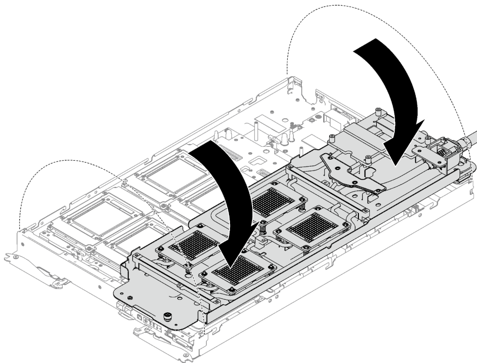
Figure 303. Plier la boucle d'eau
