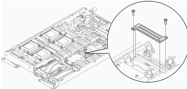
Figure 26. Retrait de la plaque de serrage VR
