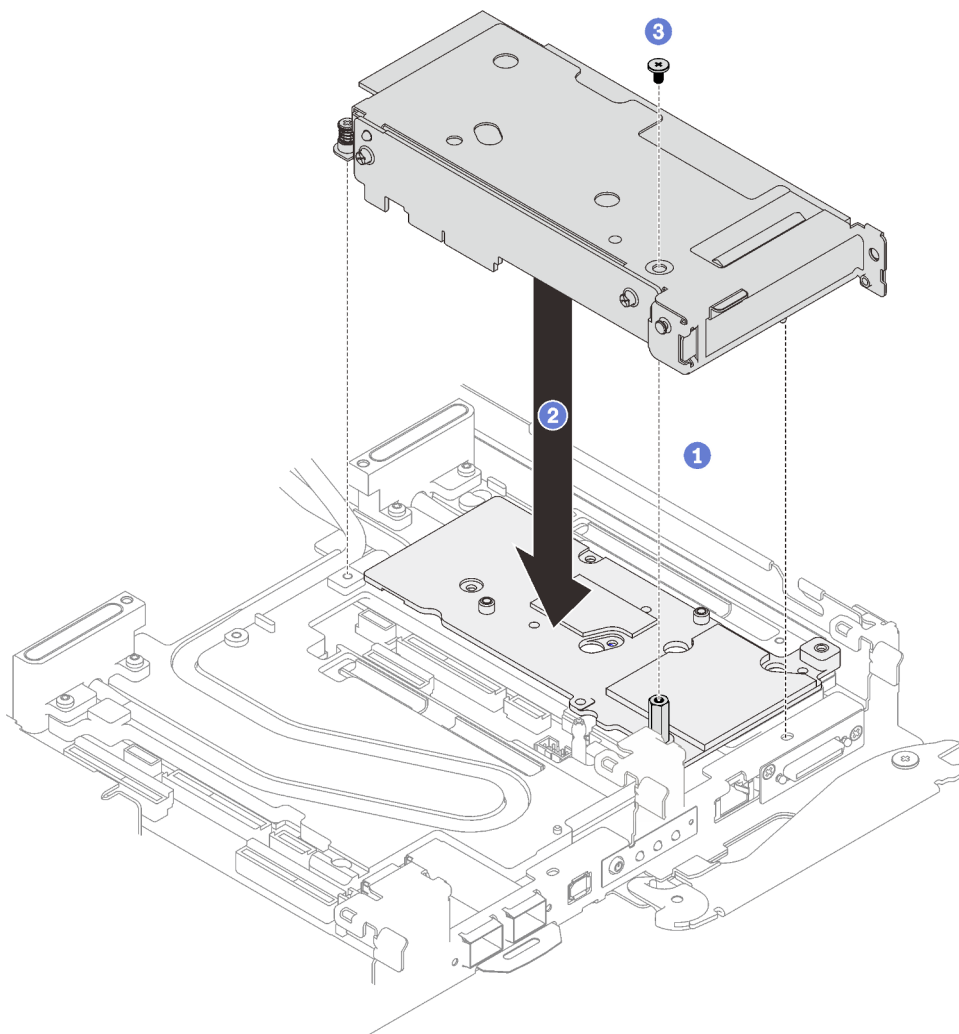
Figure 188. Installation de l'assemblage de cartes mezzanines PCIe
