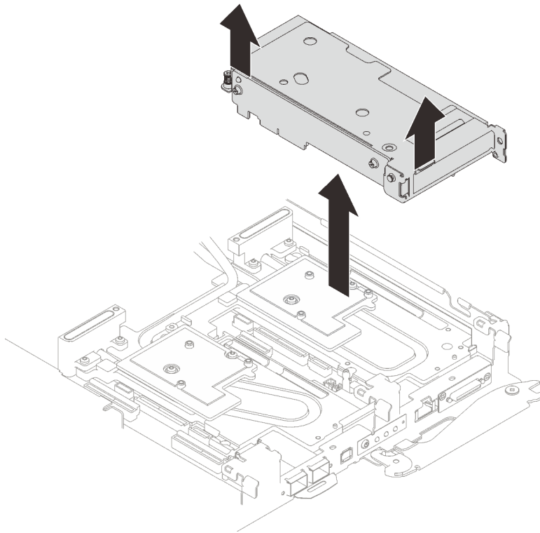
Figure 192. Retrait de l'assemblage du boîtier de cartes mezzanines PCIe
