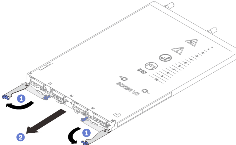
Figure 18. Retrait du plateau
