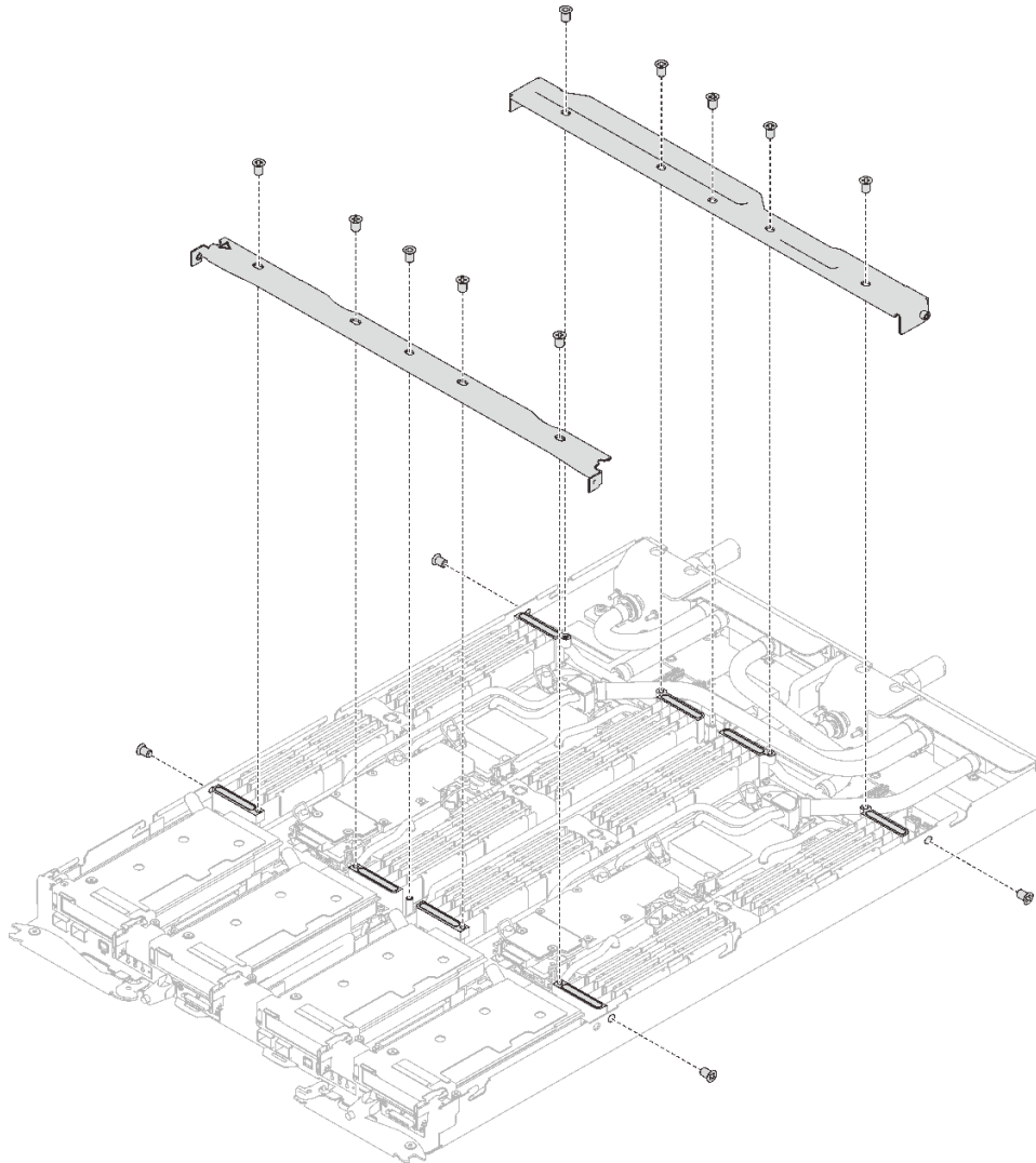
그림 21. 십자형 브레이스 설치(SD650 V3)
