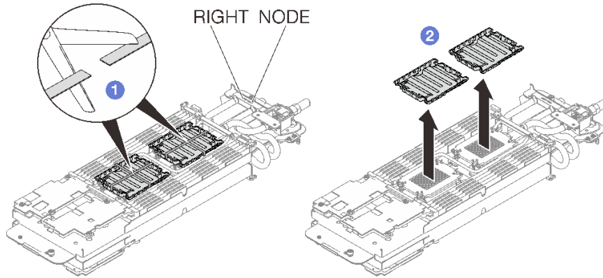
그림 39. 플라스틱 그리스 덮개 제거
