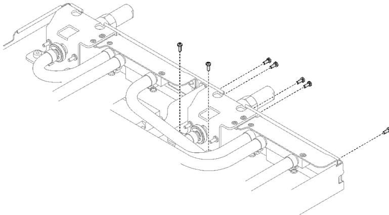
그림 191. 퀵 커넥트 나사 제거
