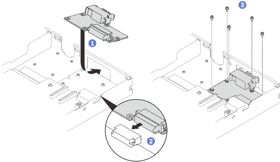
그림 197. 전원 분배 보드 설치
