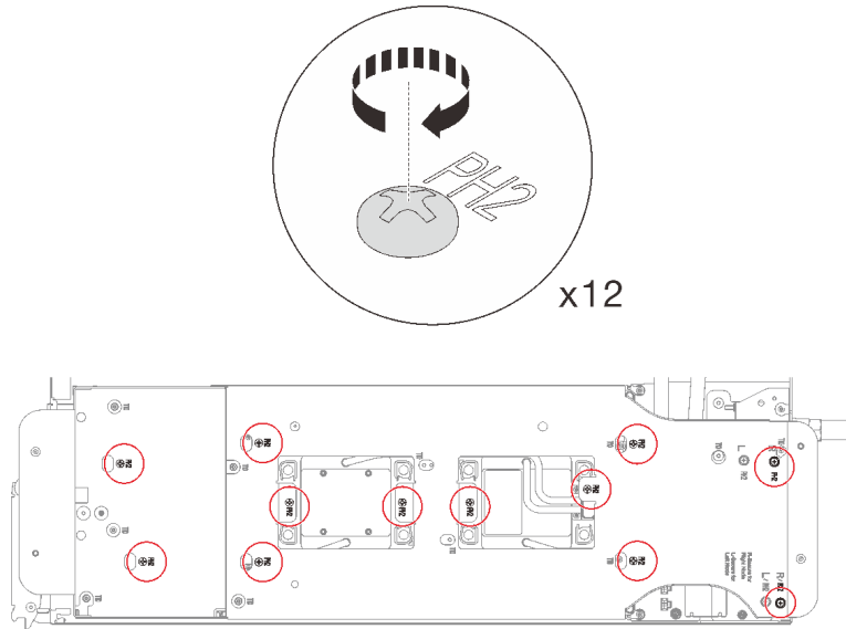
그림 193. 워터 루프 캐리어 나사 설치
