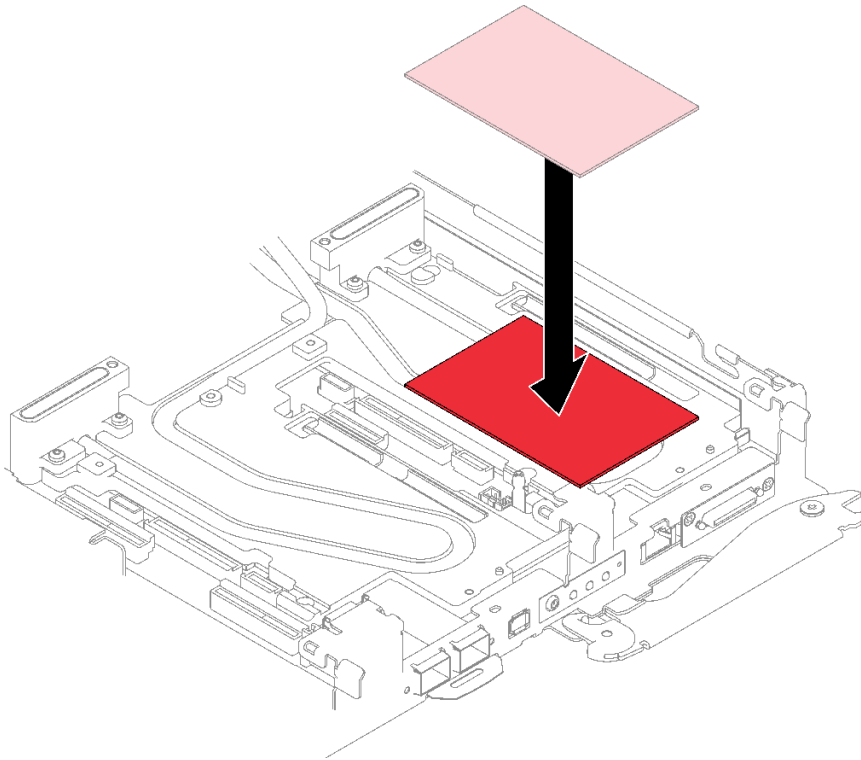
그림 118. 갭 패드 교체
