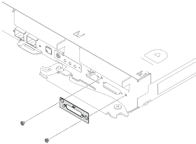
그림 122. KVM 덮개 설치
