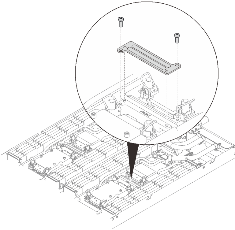
그림 189. VR 클램프판 제거
