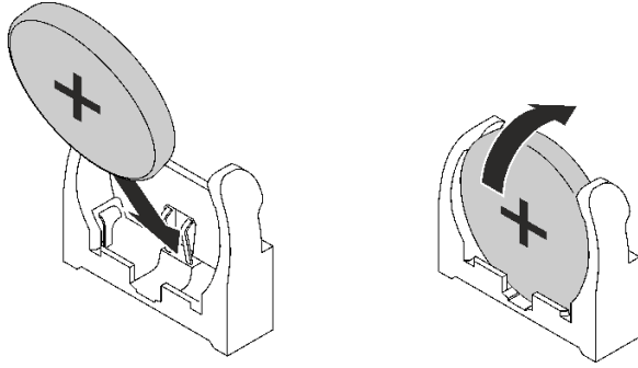
그림 55. CMOS 배터리 설치
