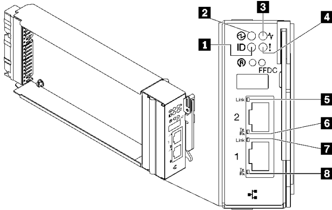
그림 253. SMM2 LED
