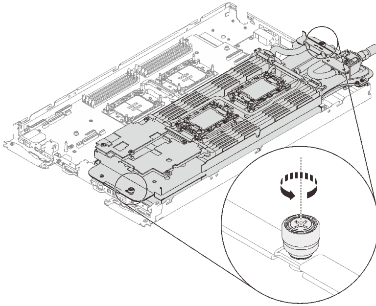
그림 44. 고정 나비 나사 풀기
