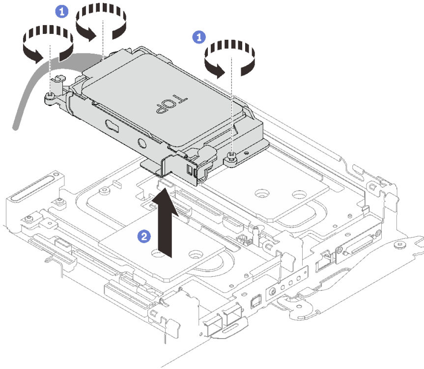
그림 63. 7mm 드라이브 케이지 어셈블리 2개 제거
