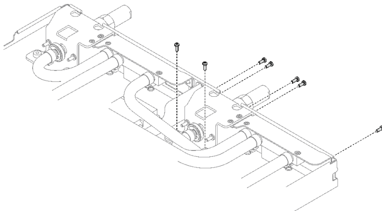
그림 204. 퀵 커넥트 나사 설치
