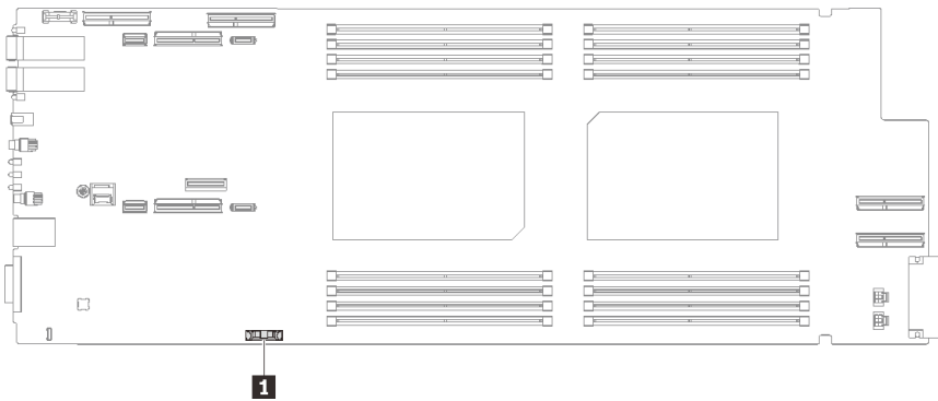
그림 54. CMOS 배터리 위치
