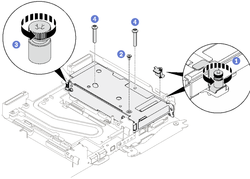
그림 163. 클램프 브래킷 고정 나사 제거
