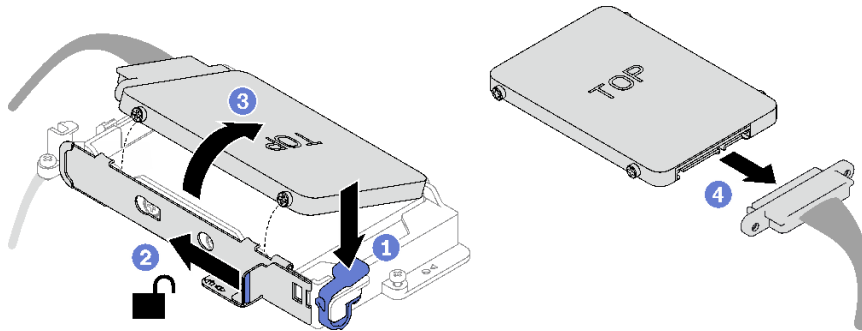
그림 67. 상단 드라이브 제거
