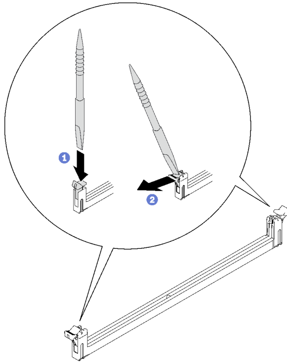
그림 136. 메모리 모듈 커넥터의 고정 클립 누르기
