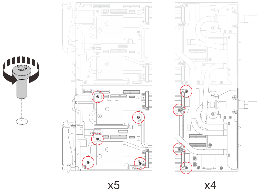
그림 208. 워터 루프 나사 제거
