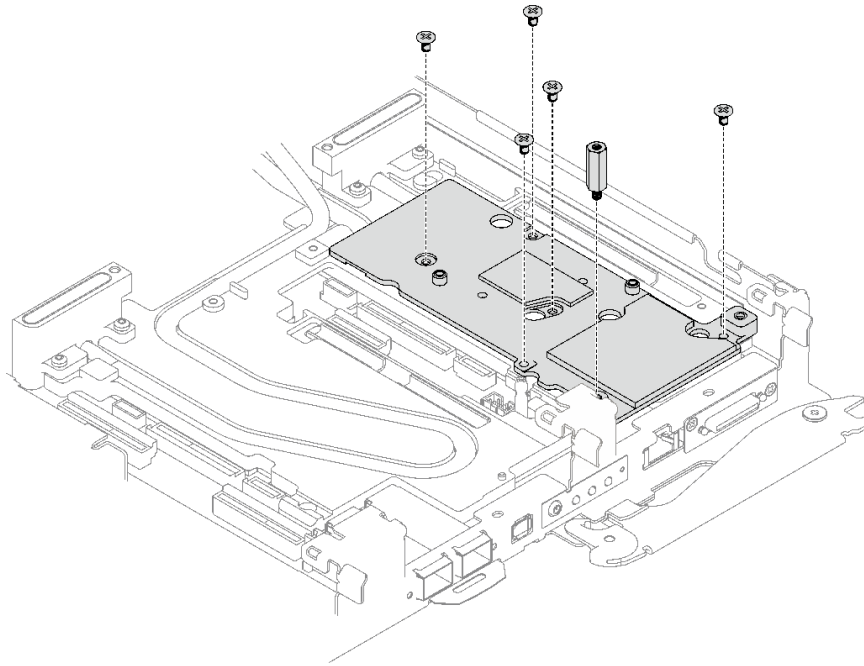
그림 165. 인터페이스판 제거
