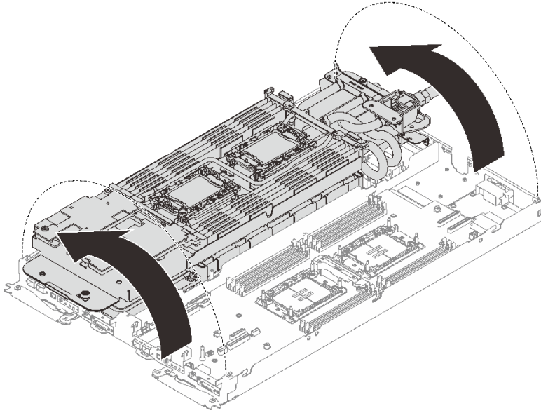
그림 28. 워터 루프 접기
