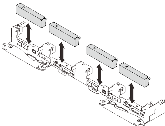
그림 116. 빈 베젤 필터 설치
