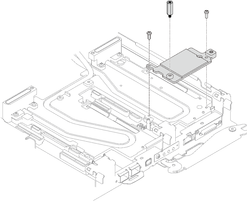
그림 154. 인터페이스판 제거
