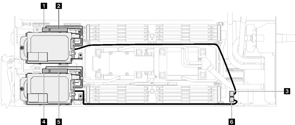
그림 120. E3.S 드라이브 케이블 배선
