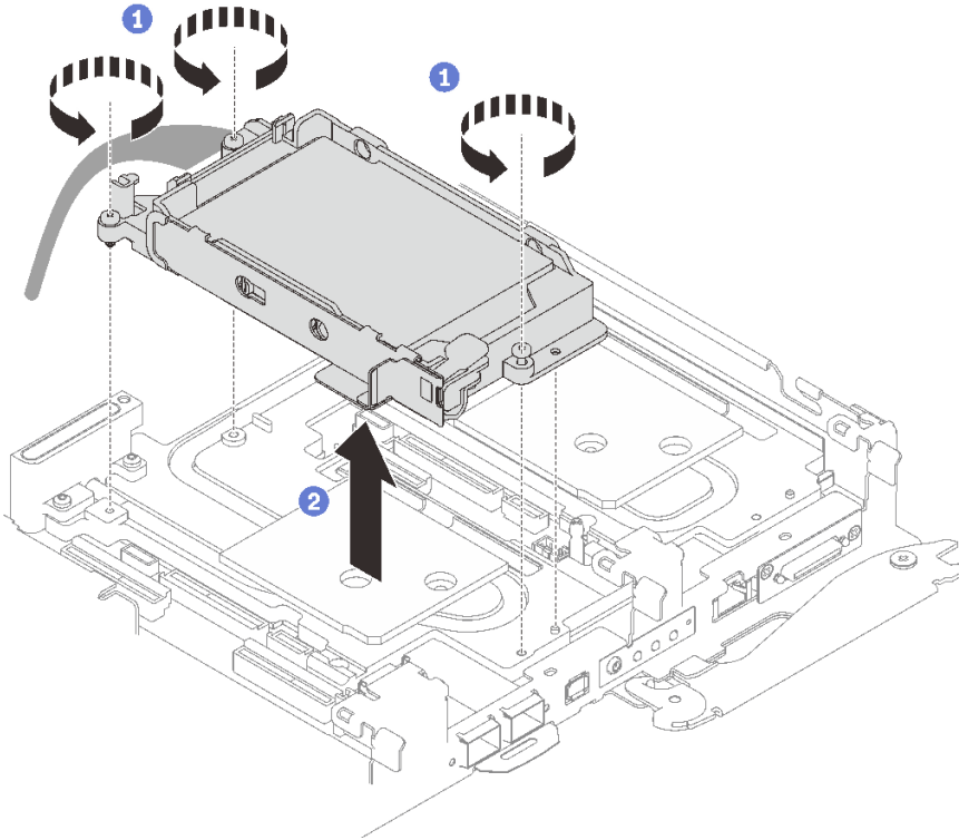
그림 61. 15mm 드라이브 케이지 어셈블리 1개 제거
