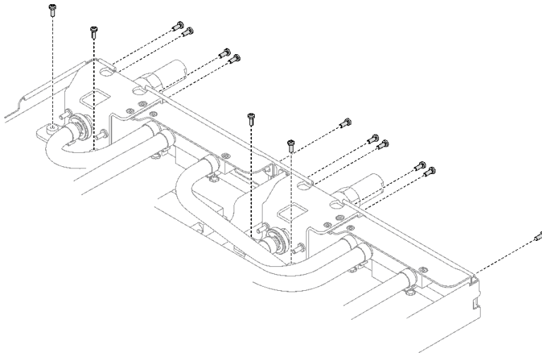
그림 50. 퀵 커넥트 나사 설치
