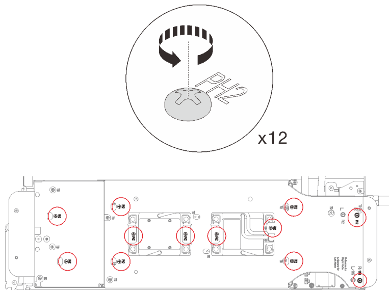
그림 201. 워터 루프 캐리어 나사 풀기
