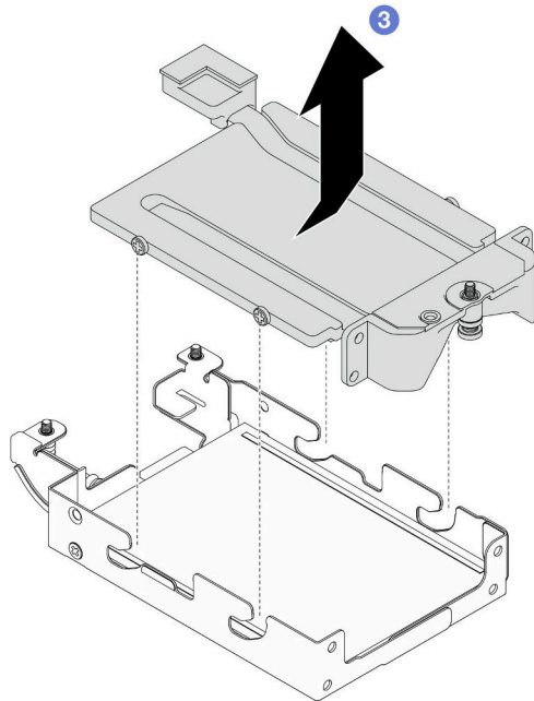
그림 106. 전도판 제거
