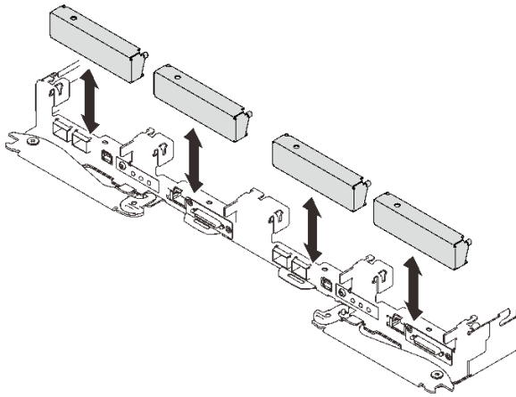
그림 64. 빈 베젤 필터 제거
