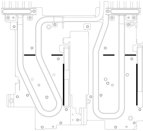
그림 117. E3.S 갭 패드를 맞추기 위한 워터 루프의 표시
