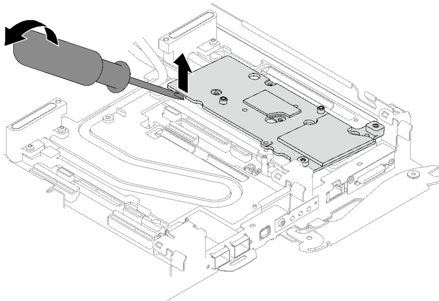
그림 167. 워터 루프 냉각판에서 인터페이스판 분리
