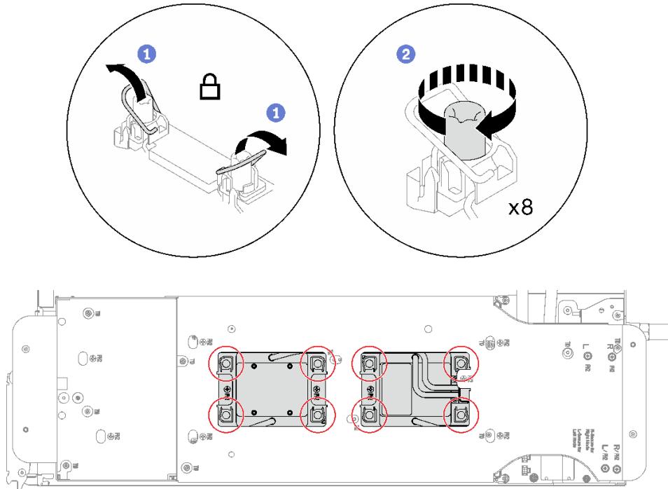
그림 227. 프로세서 설치
