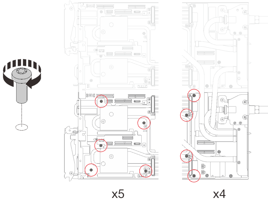
그림 203. 워터 루프 나사 설치
