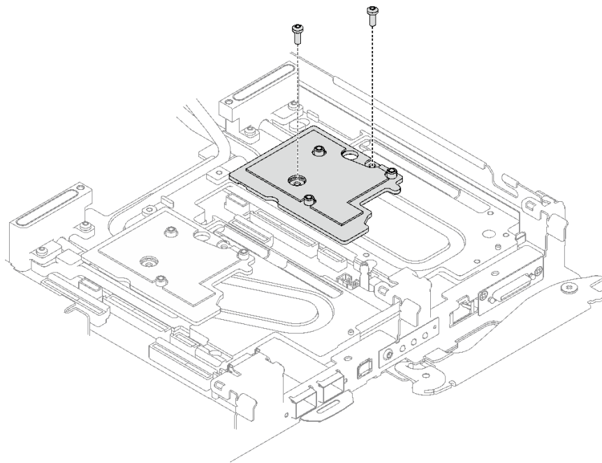
그림 179. 인터페이스판 제거
