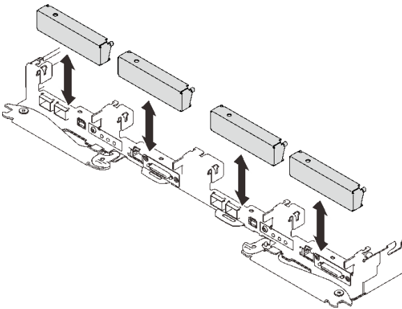
그림 155. 빈 베젤 필터 설치
