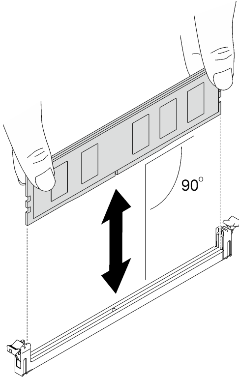
그림 142. 메모리 모듈 설치
