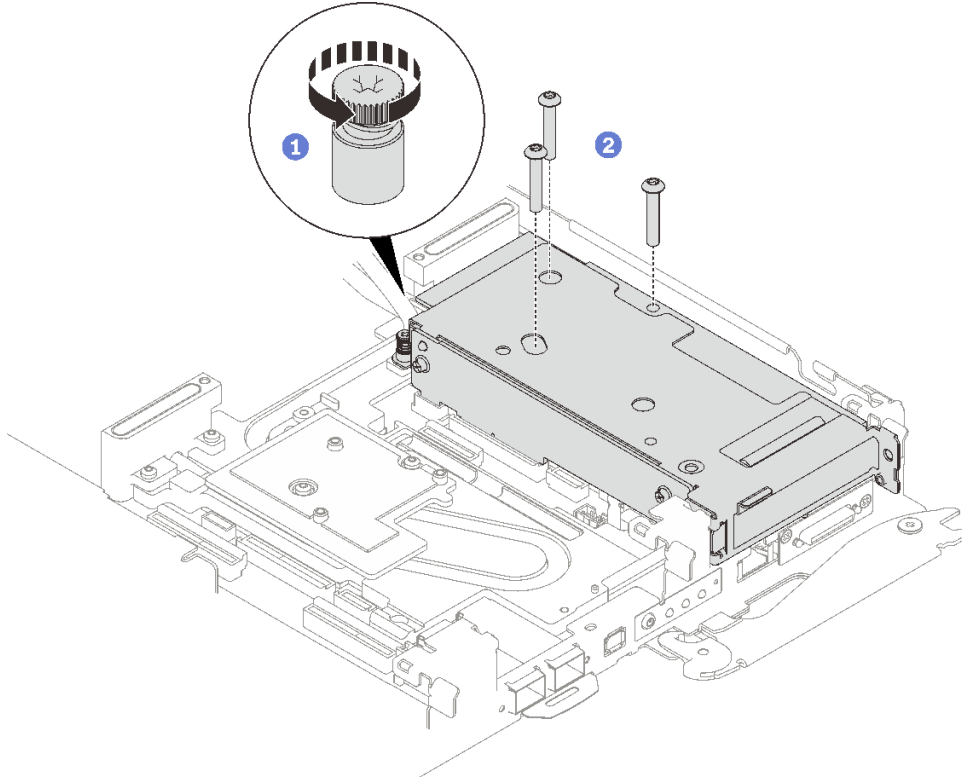
그림 176. PCIe 라이저 어셈블리 제거
