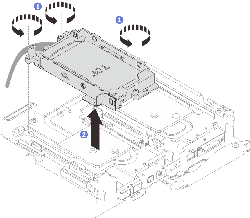
그림 62. 7mm 드라이브 케이지 어셈블리 1개 제거
