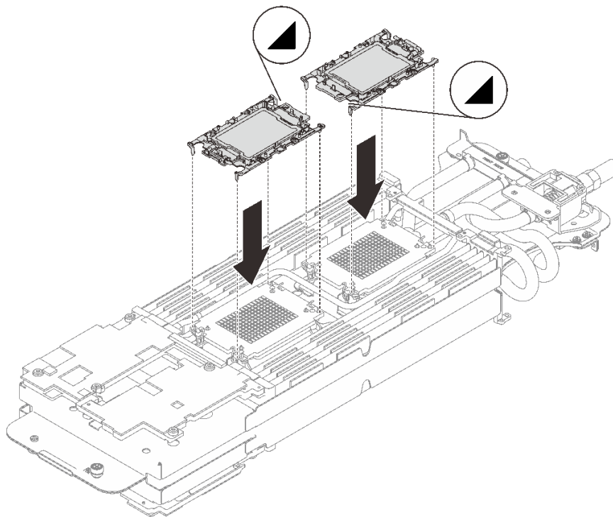
그림 40. 프로세서 설치
