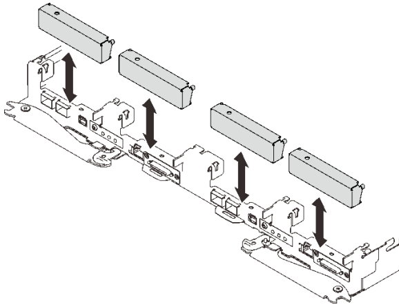
그림 169. 빈 베젤 필터 설치
