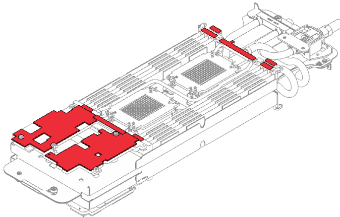
그림 225. 워터 루프 갭 패드
