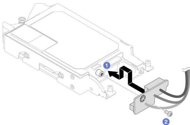
그림 113. E3.S 케이블 종단 백플레인 설치
