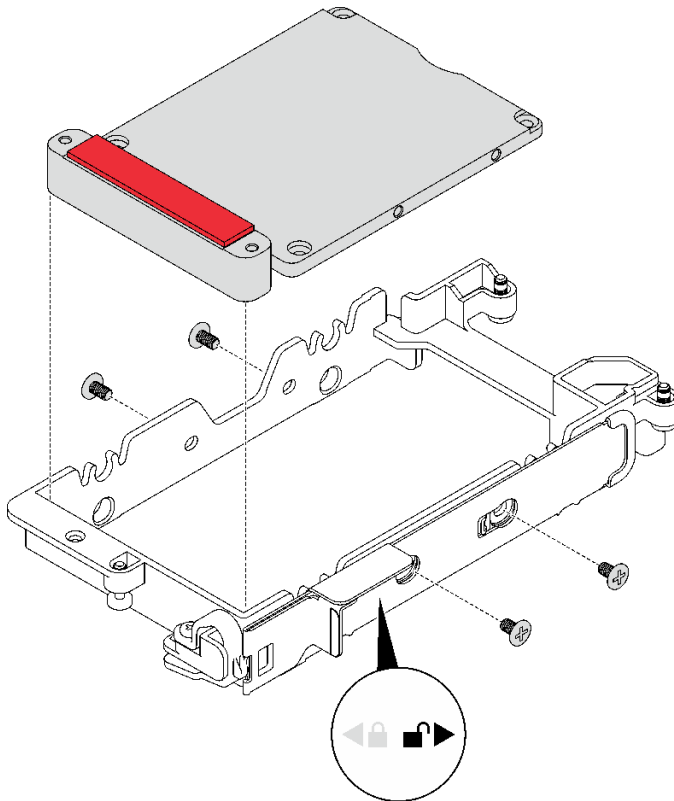
그림 69. 전도판 제거
