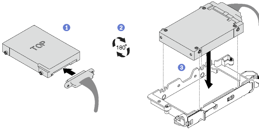
그림 71. 15mm 드라이브 설치
