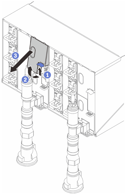
그림 260. 상단 EMC 실드 제거
