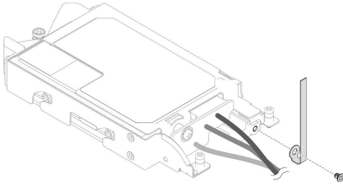
그림 114. 케이블 타이 설치
