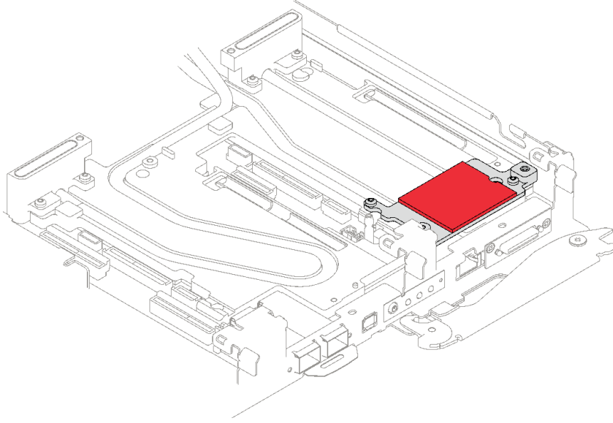
그림 159. CX-6 라이저용 인터페이스판 퍼티 패드
