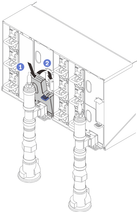
그림 262. 하단 EMC 실드 설치
