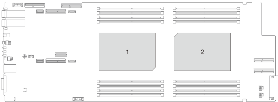
그림 217. 프로세서 위치
