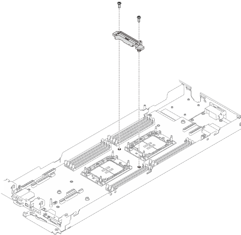
그림 233. VR 워터 루프 홈 제거
