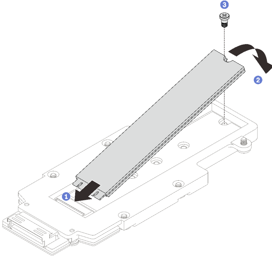
그림 133. M.2 드라이브 설치
