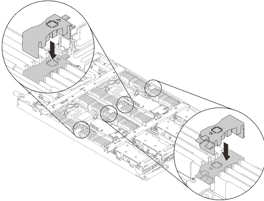
그림 58. DIMM 콤 설치
