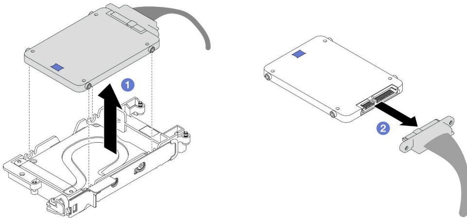
그림 88. 하단 드라이브 제거
