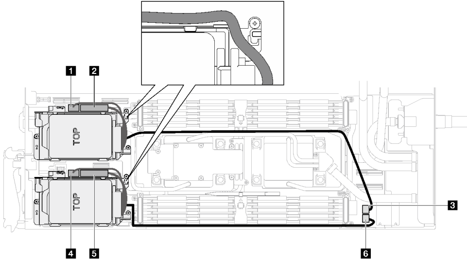
그림 60. 드라이브 어셈블리 케이블 배선
