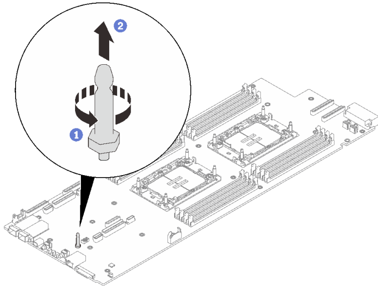
그림 236. 가이드 핀 제거
