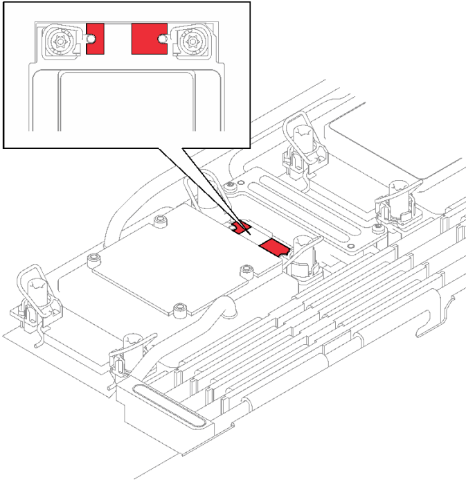
그림 127. 프로세서 냉각판의 갭 패드
