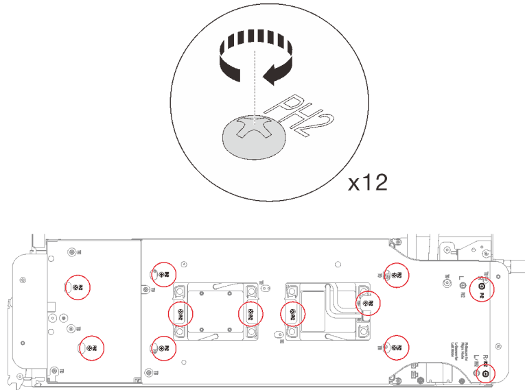
그림 211. 워터 루프 캐리어 나사 설치
