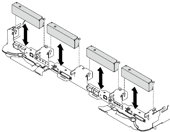
그림 86. 빈 베젤 필러 제거
