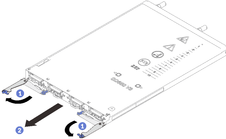
그림 16. 트레이 제거
