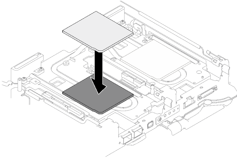
그림 95. 갭 패드 교체
