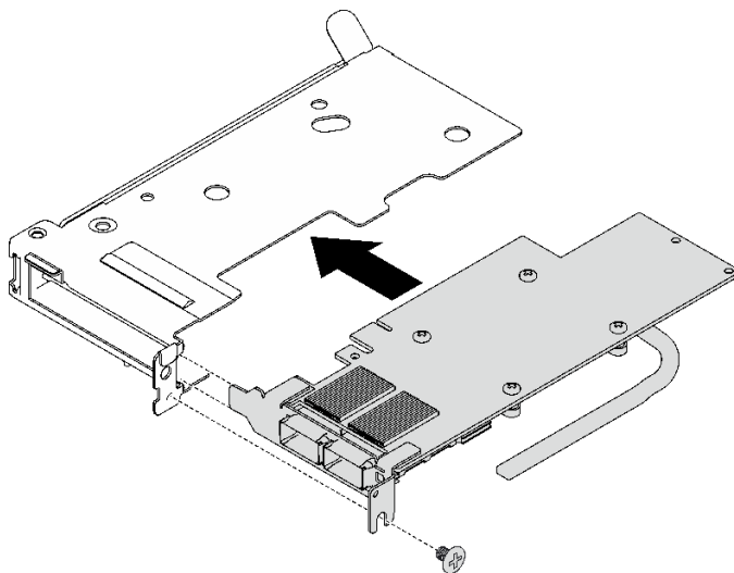
그림 150. PCIe 어댑터 설치
