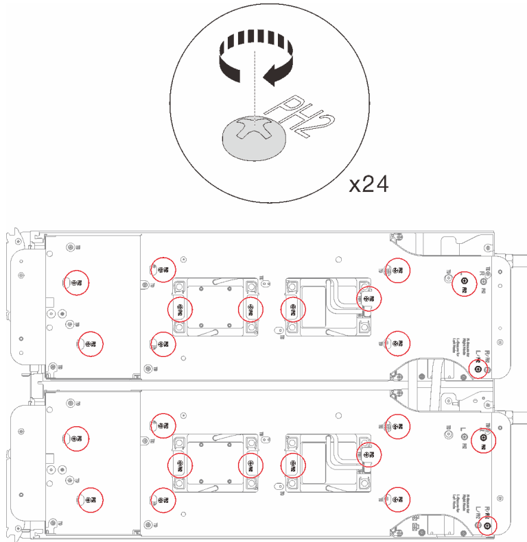
그림 26. 워터 루프 캐리어 나사 설치
