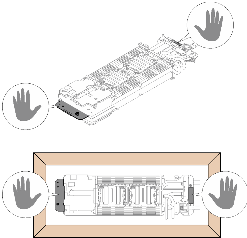
그림 38. 패키지 박스에서 워터 루프를 제거할 때의 터치 포인트
