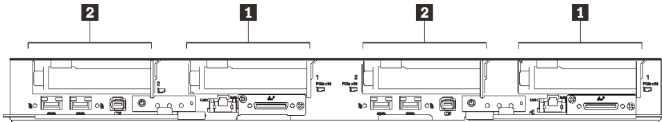
그림 8. PCIe 슬롯 번호 - SD650 V3 트레이
