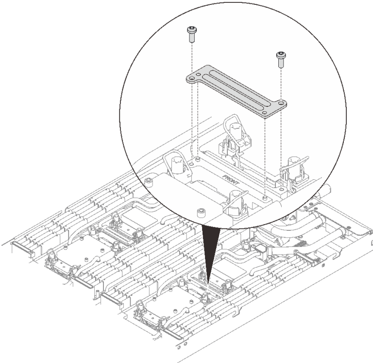
그림 22. VR 클램프판 제거
