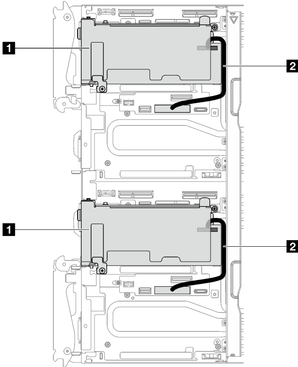
그림 243. ConnectX-7 NDR 200/ConnectX-7 NDR 400 케이블 배선에 대한 소켓 직접 구성
