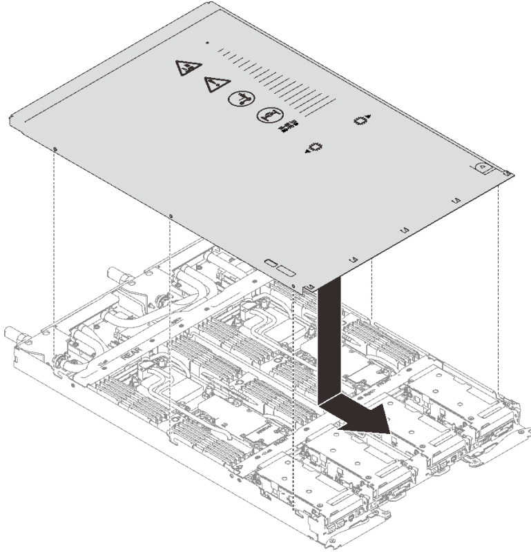
그림 19. 트레이 덮개 설치
