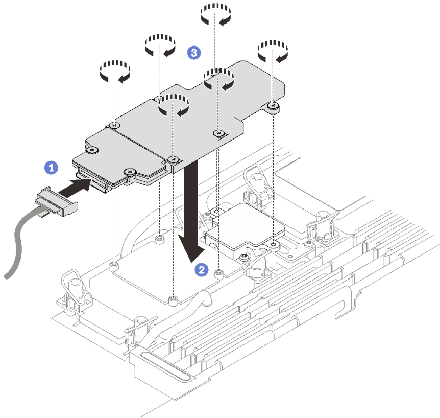
그림 129. M.2 백플레인 어셈블리 설치
