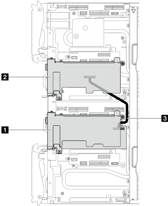
그림 241. ConnectX-6 케이블 배선에 대한 공유 I/O 구성
