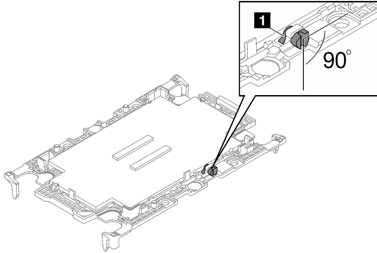
그림 221. 프로세서 고정장치의 TIM 차단 캠
