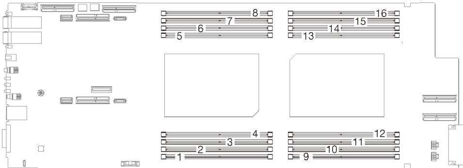
그림 134. 메모리 모듈 커넥터 위치
