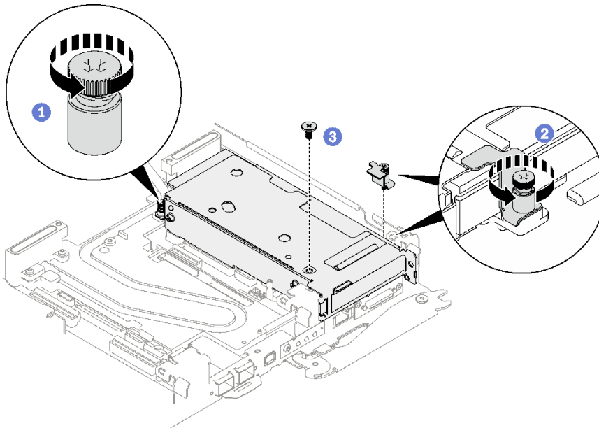
그림 152. 클램프 브래킷 고정 나사 제거
