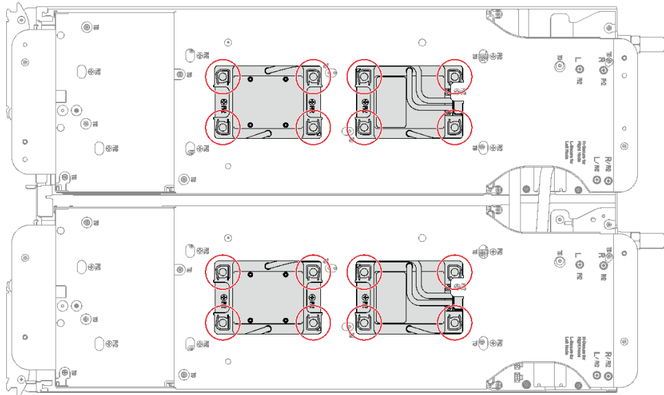
그림 27. Torx T30 고정 나사 풀기
