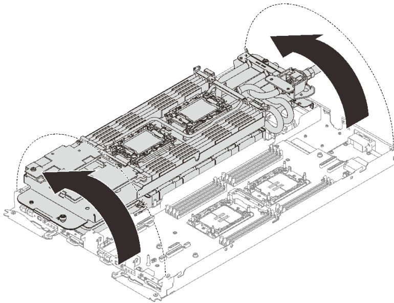
그림 213. 워터 루프 접기
