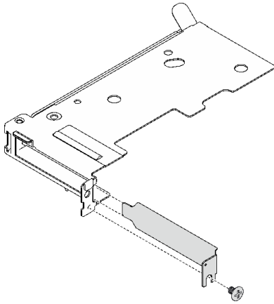
그림 148. 필터 제거
