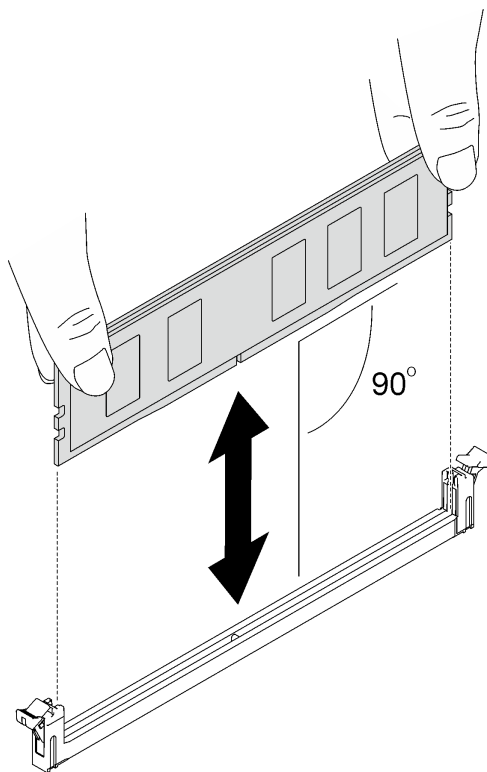
그림 137. 메모리 모듈 제거
