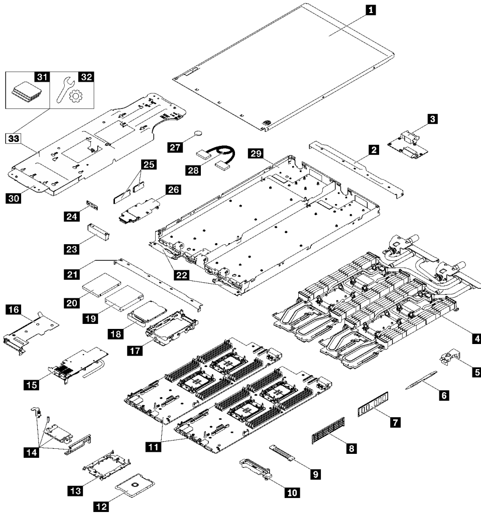
그림 9. SD650 V3 부품 목록
