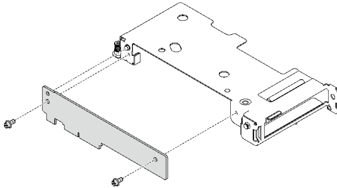
그림 156. 확장 보드 제거
