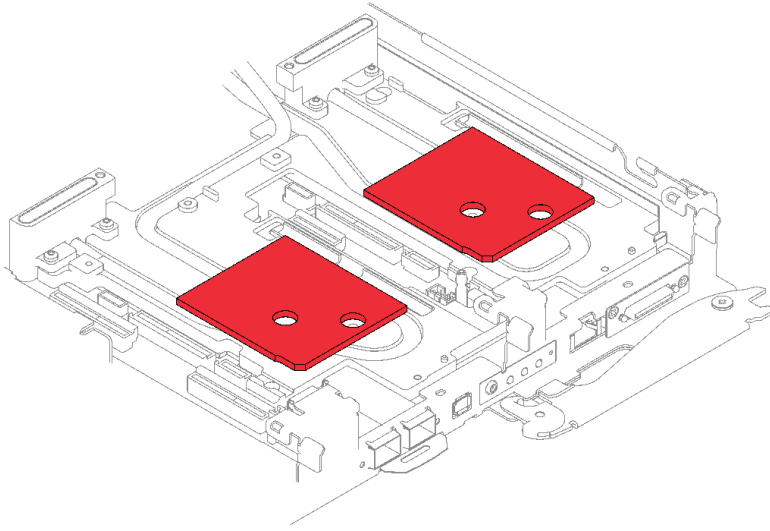
그림 79. 캡 패드 위치
