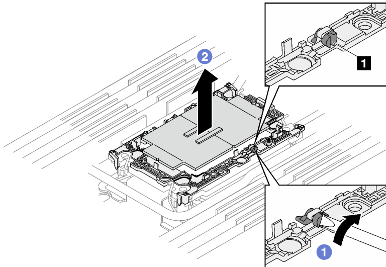
그림 215. 프로세서 제거(Intel® Xeon® CPU Max 프로세서)
