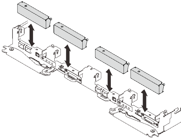
그림 157. 빈 베젤 필터 제거
