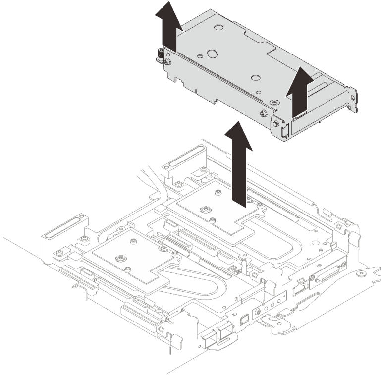
그림 178. PCIe 라이저 케이지 어셈블리 제거
