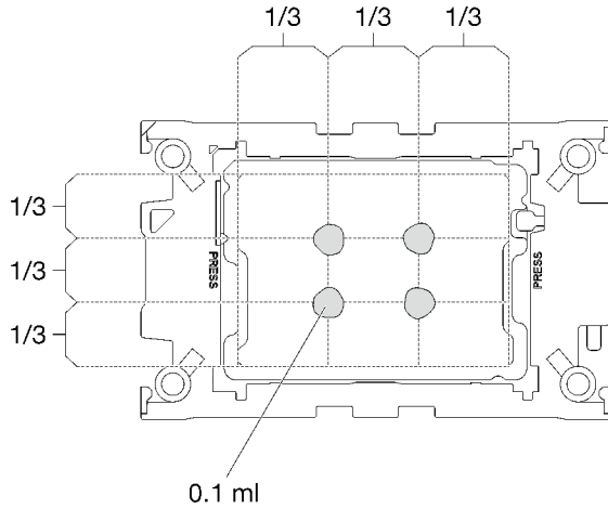
그림 218. 열전도 그리스 도포
