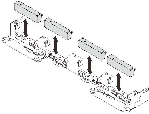
그림 183. 빈 베젤 필러 설치
