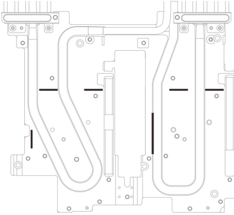
그림 77. 갭 패드를 맞추기 위한 워터 루프의 표시
