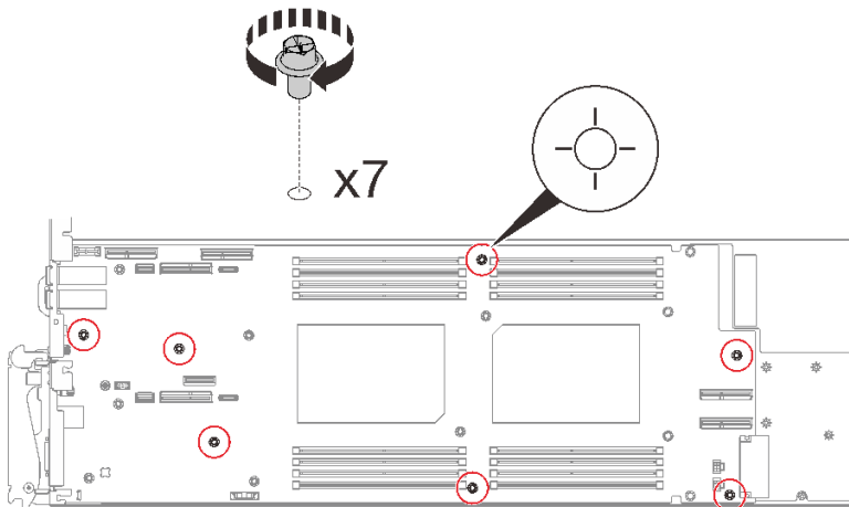
그림 238. 시스템 보드 나사 설치
