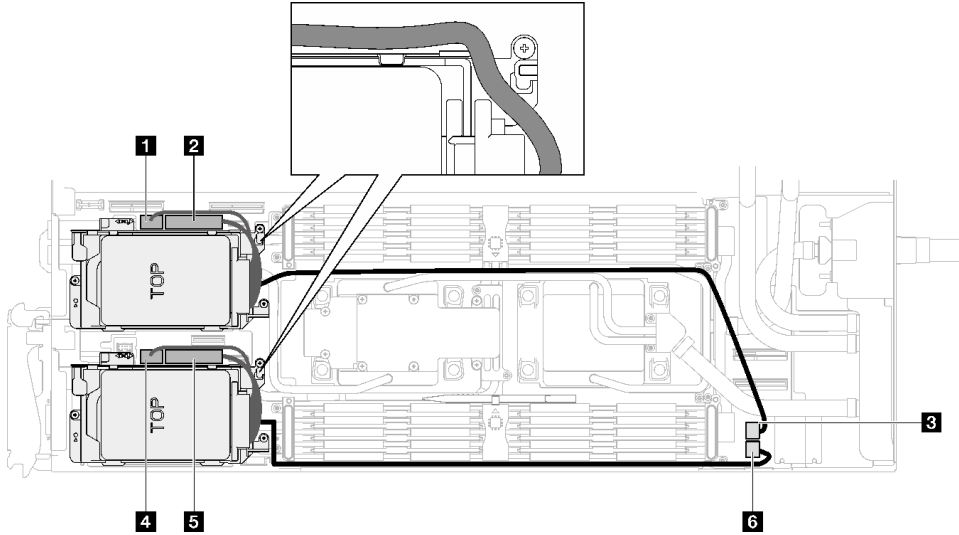
그림 98. 드라이브 어셈블리 케이블 배선
