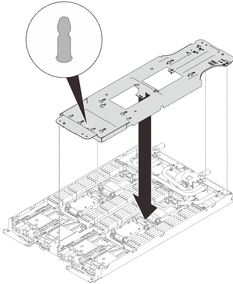
그림 192. 워터 루프 캐리어 설치
