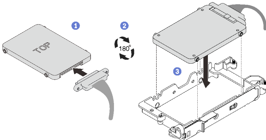
그림 73. 아래쪽 드라이브 설치
