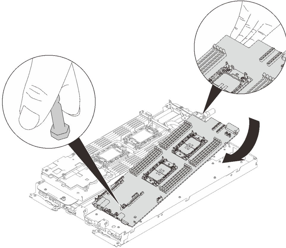
그림 237. 시스템 보드 설치
