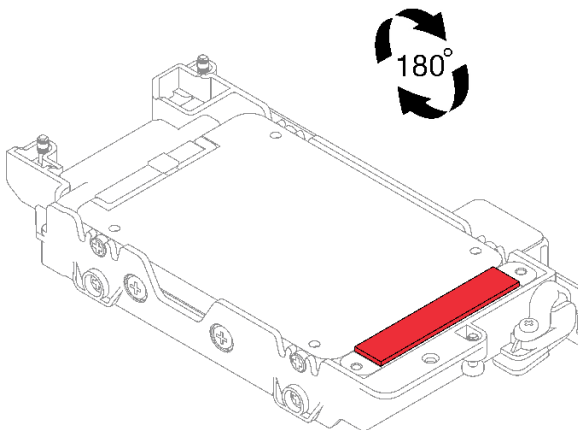
그림 76. 갭 패드 위치
