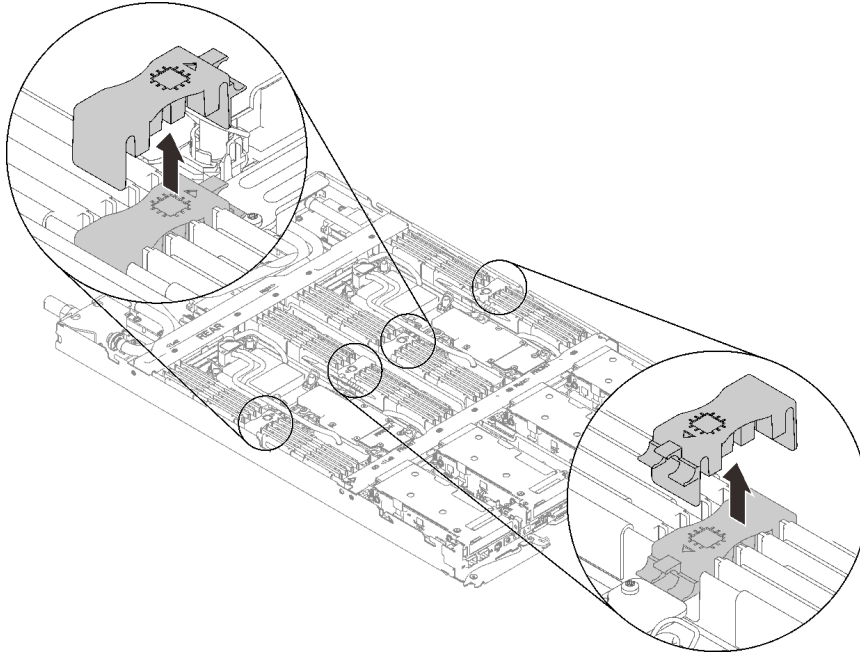
그림 57. DIMM 콤 제거
