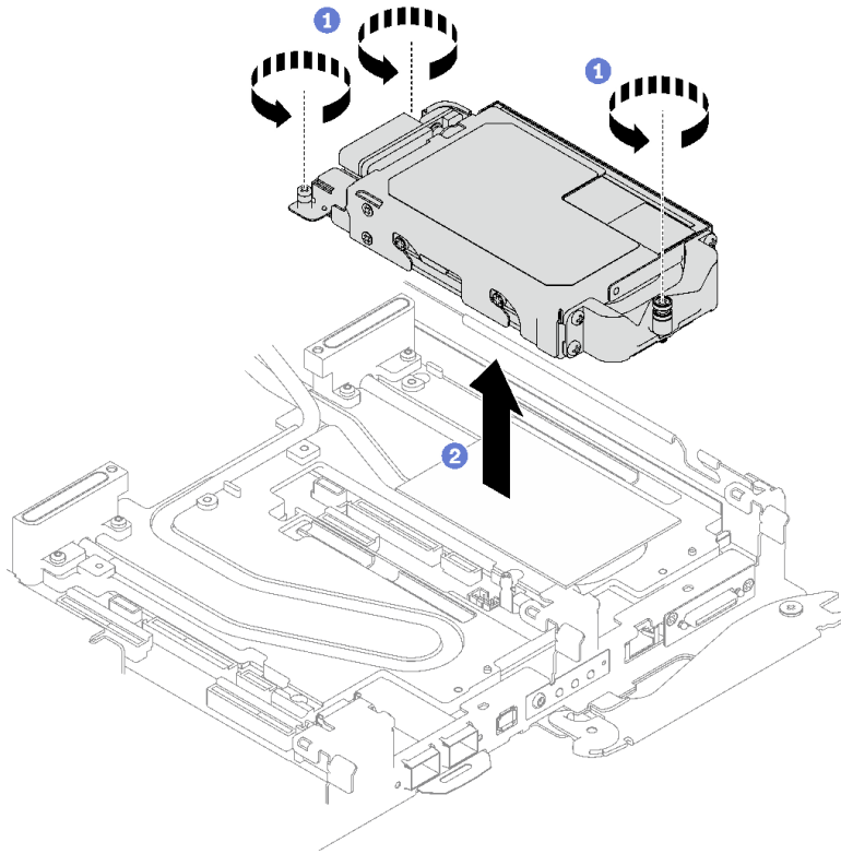
그림 100. E3.S 드라이브 케이지 어셈블리 제거
