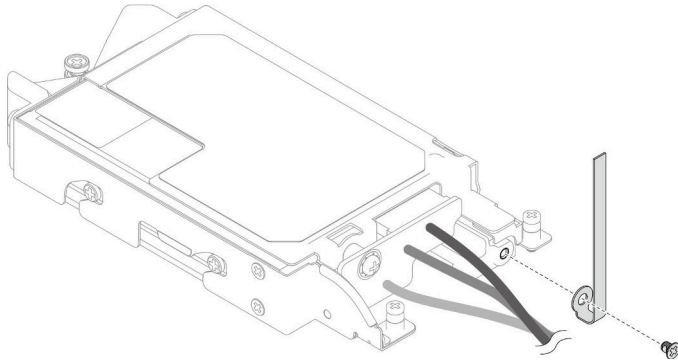
그림 103. 케이블 타이 제거
