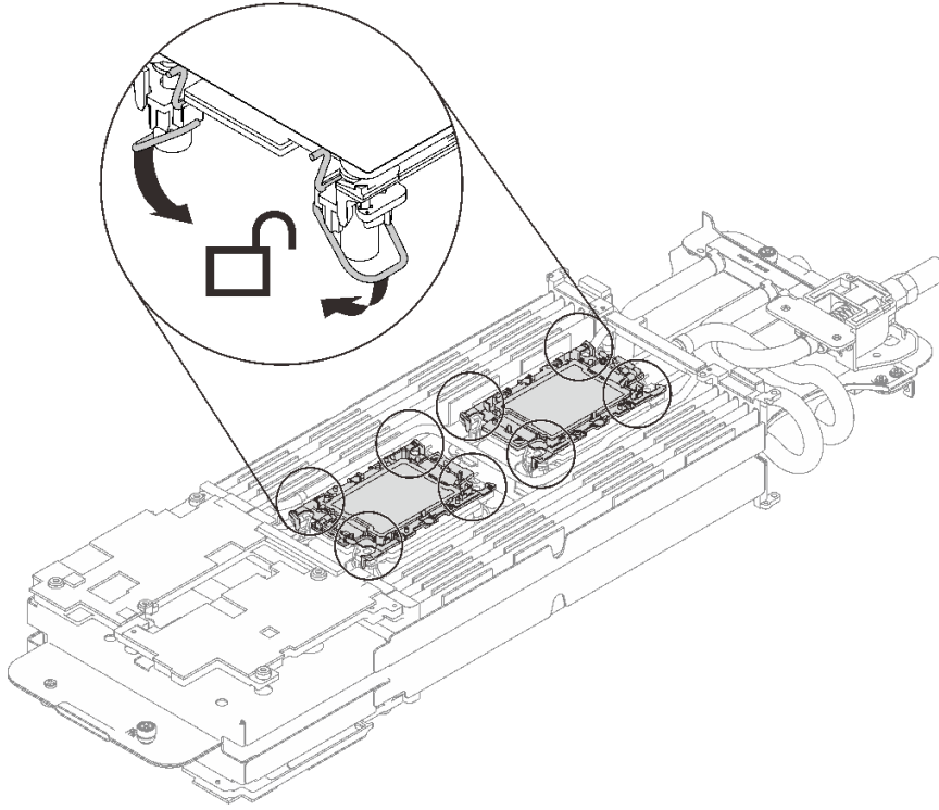
그림 224. 프로세서 잠금 해제 위치
