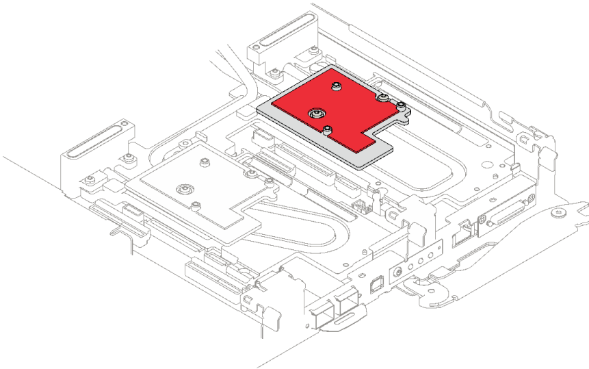
그림 187. CX-7 NDR 400용 인터페이스판의 갭 패드
