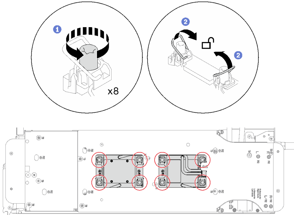
그림 212. 프로세서 풀기
