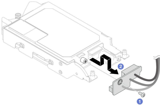
그림 104. E3.S 드라이브 케이블 중단 백플레인 제거
