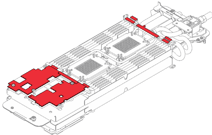
그림 42. 워터 루프 갭 패드
