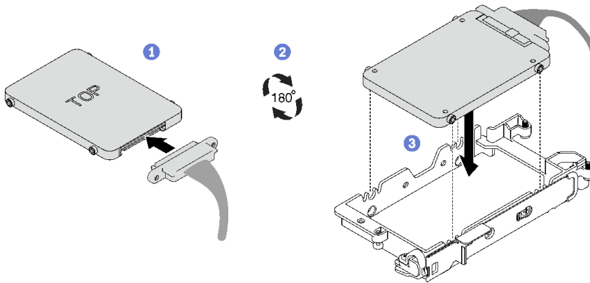
그림 70. 7mm 드라이브 설치
