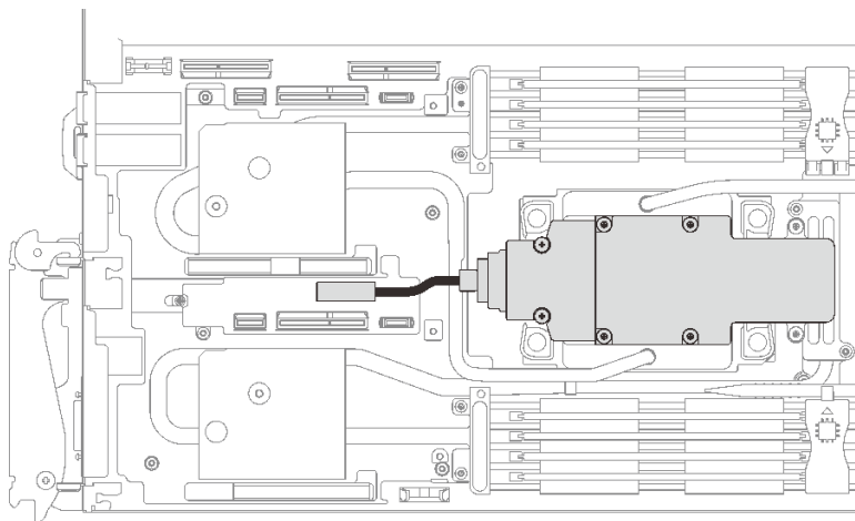
그림 130. M.2 백플레인 어셈블리 케이블 설치
