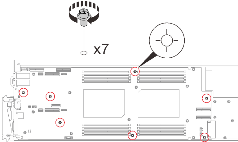
그림 234. 시스템 보드 나사 제거
