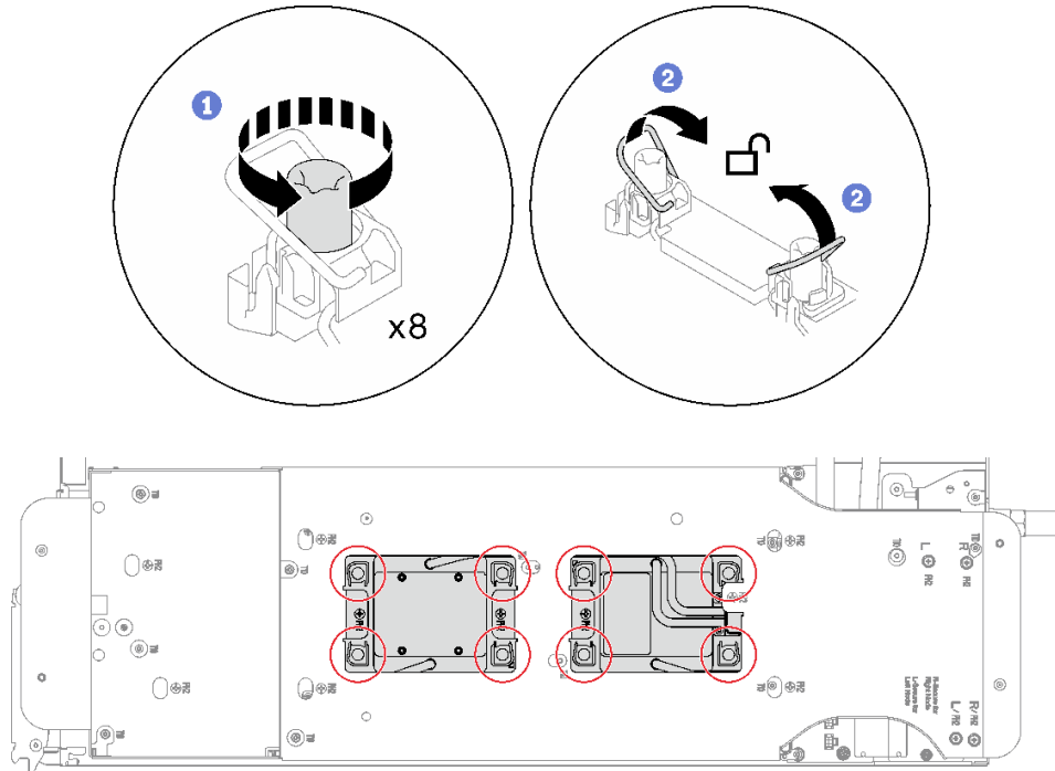
그림 194. 프로세서 풀기
