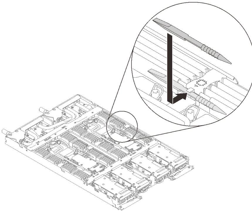
그림 144. 메모리 모듈 도구 설치
