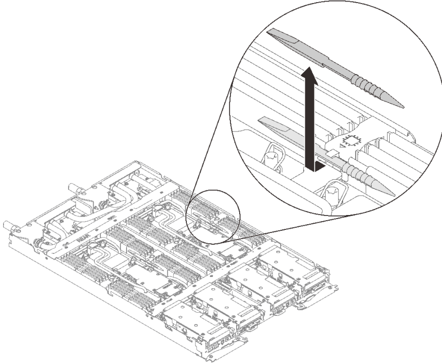
그림 56. 메모리 모듈 도구 제거
