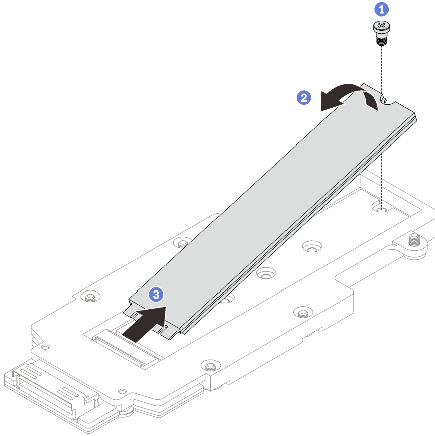
그림 131. M.2 드라이브 제거
