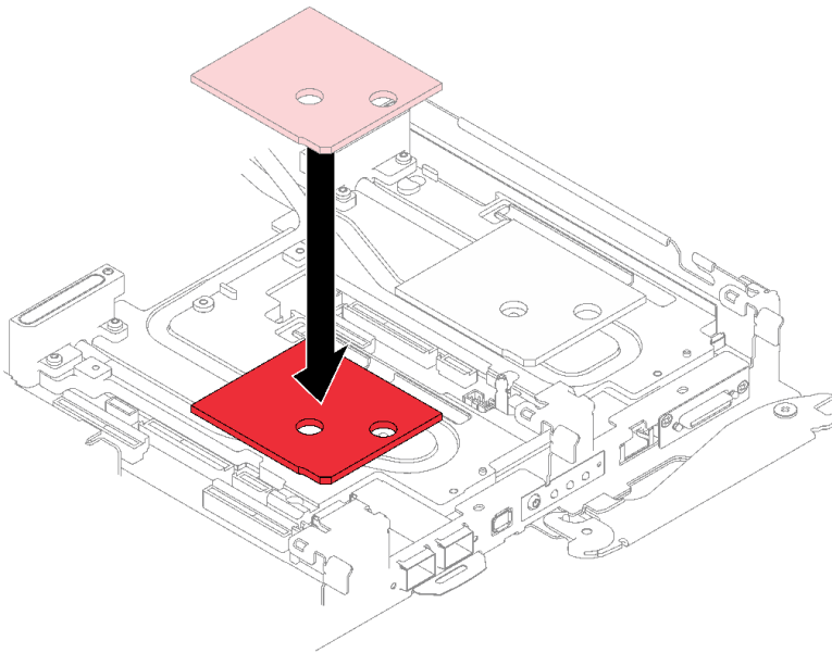
그림 78. 갭 패드 교체
