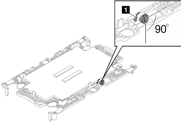
그림 37. 프로세서 고정장치의 TIM 차단 캠
