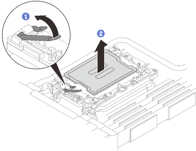
그림 214. 프로세서 제거
