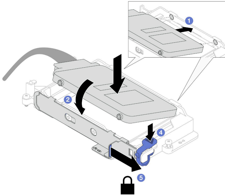
그림 92. 위쪽 드라이브 설치
