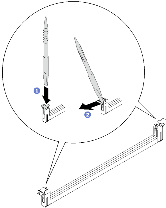
그림 141. 메모리 모듈 커넥터의 고정 클립 누르기
