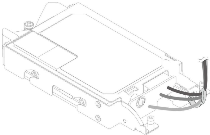
그림 115. 케이블 타이로 케이블 묶기
