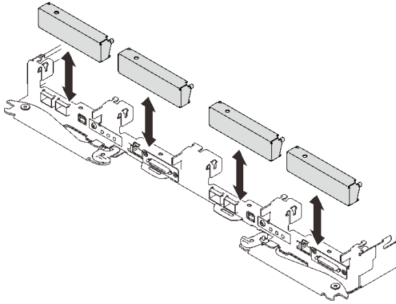
그림 171. 빈 베젤 필터 제거
