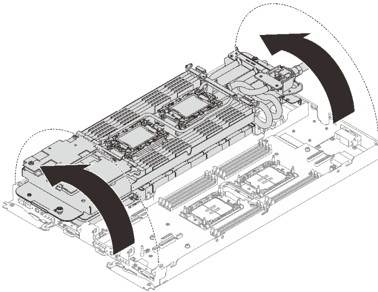
그림 195. 워터 루프 접기
