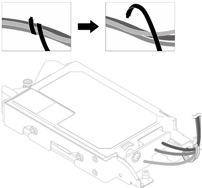
그림 102. 케이블 타이에서 케이블 분리
