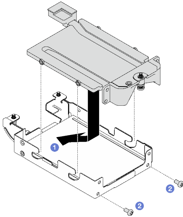
그림 111. E3.S 드라이브 전도판 설치
