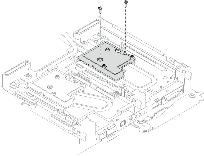
그림 186. 인터페이스판 설치
