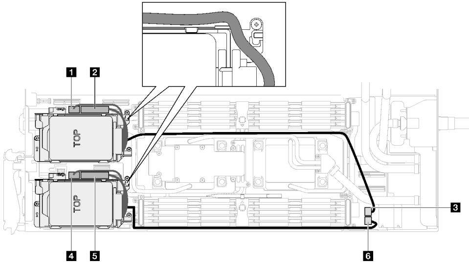
그림 83. 드라이브 어셈블리 케이블 배선
