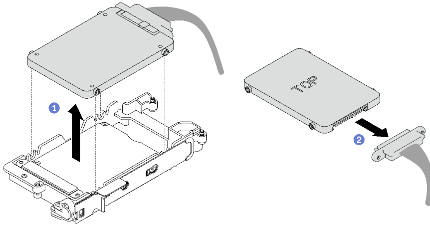
그림 68. 하단 드라이브 제거
