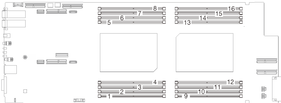
그림 6. 컴퓨팅 노드 시스템 보드의 DIMM 슬롯 번호
