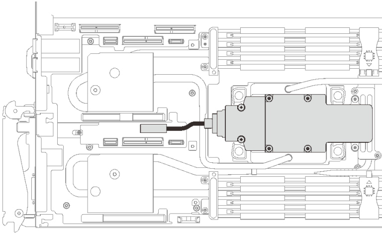
그림 123. M.2 백플레인 어셈블리 케이블 제거
