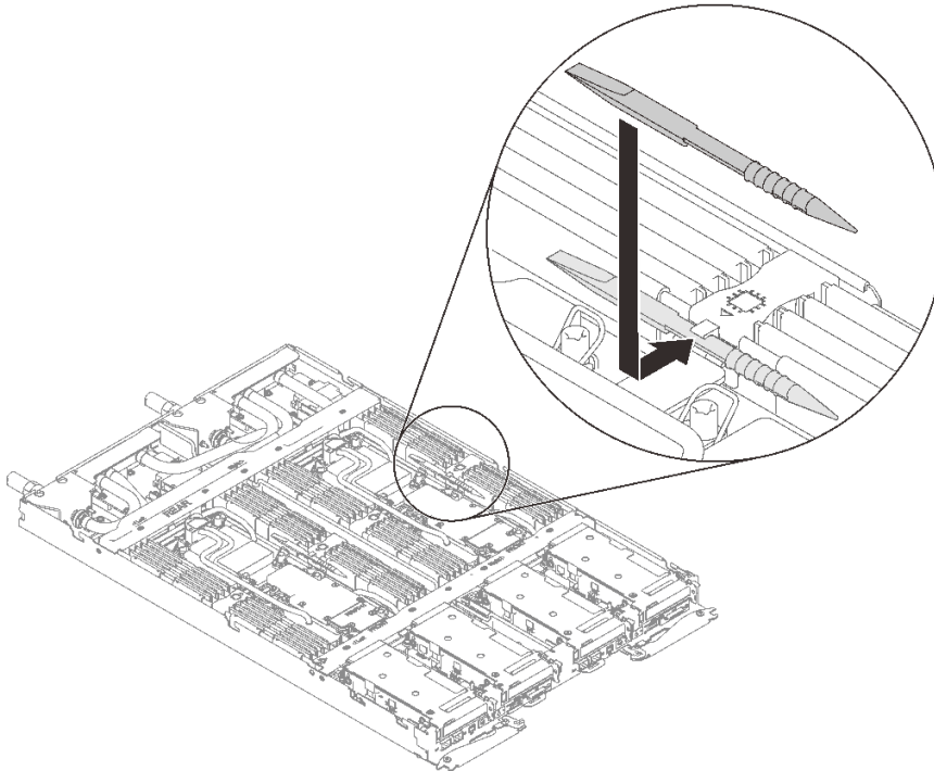
그림 59. 메모리 모듈 도구 설치
