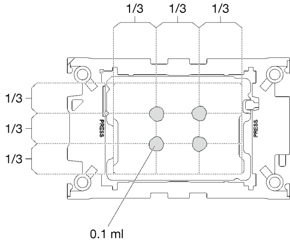
그림 34. 열전도 그리스 도포
