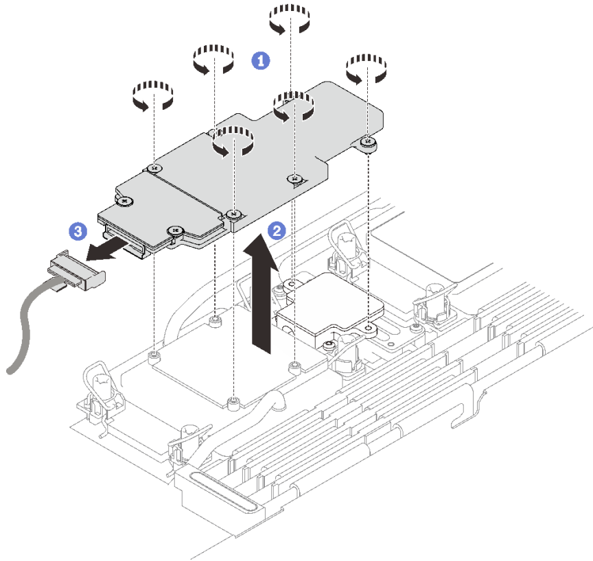
그림 124. M.2 백플레인 어셈블리 제거
