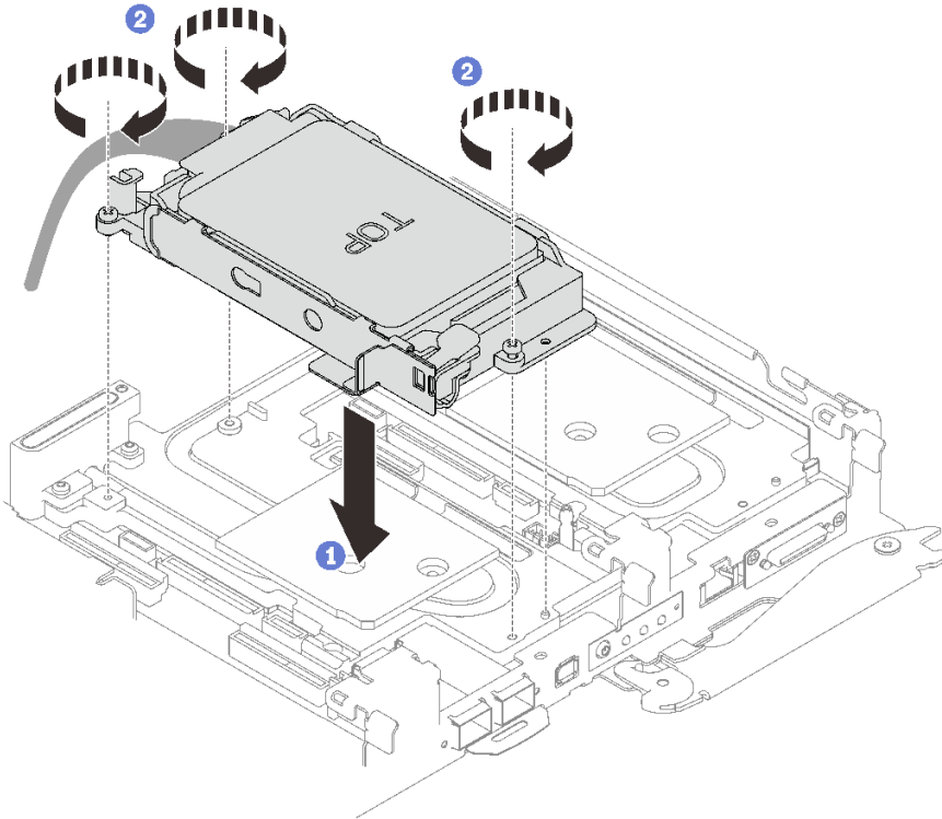
그림 82. 7mm 드라이브 케이지 어셈블리 2개 설치
