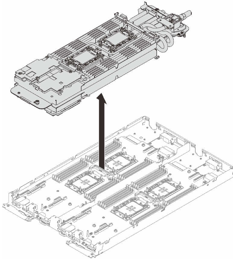
그림 33. 워터 루프 제거
