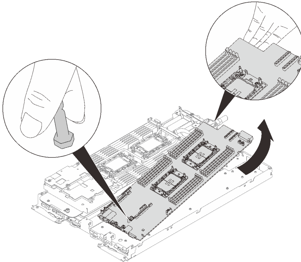
그림 235. 시스템 보드 제거
