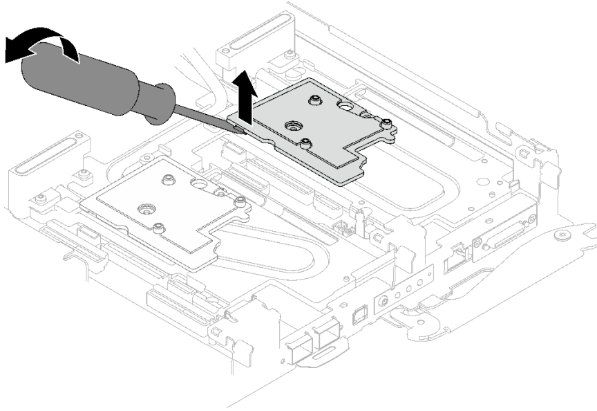
그림 181. 워터 루프 냉각판에서 인터페이스판 분리
