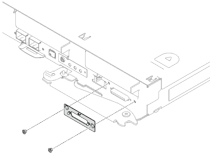
그림 121. KVM 덮개 제거
