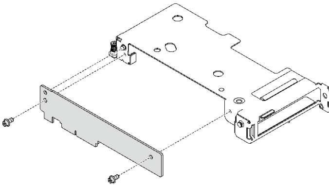
그림 184. 확장 보드 제거
