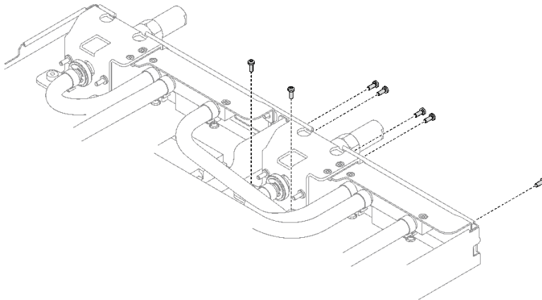
그림 209. 퀵 커넥트 나사 제거
