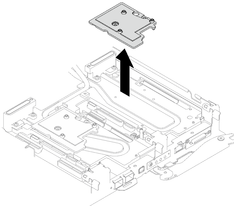
그림 182. 인터페이스판 제거
