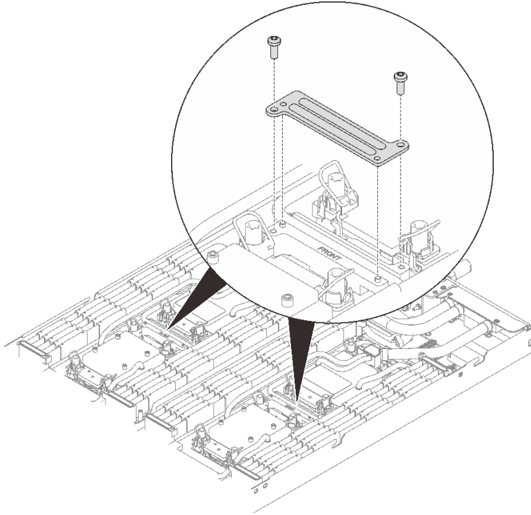
그림 51. VR 클램프판 설치
