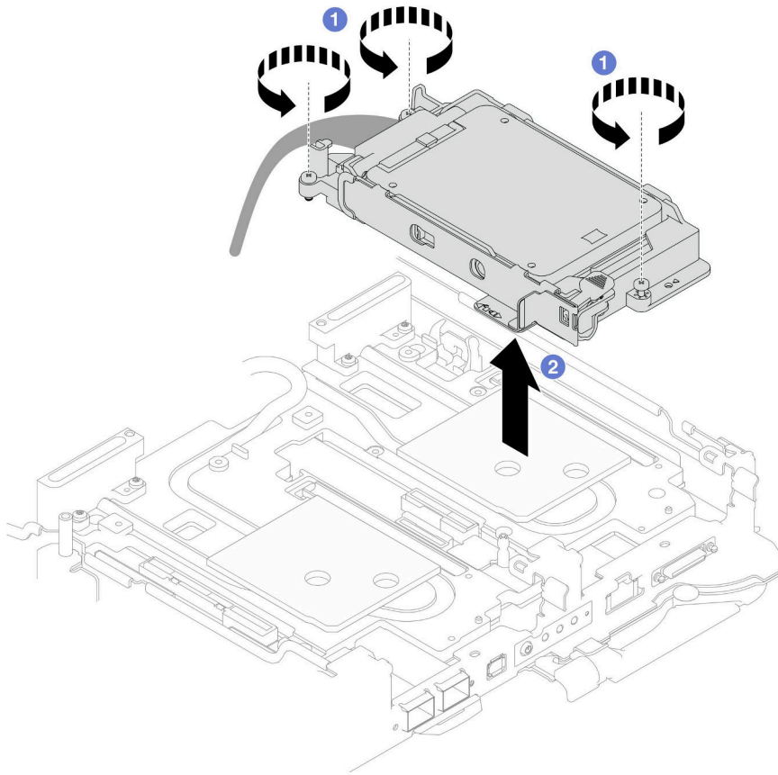
그림 85. 7mm NVMe 드라이브 케이지 어셈블리 제거
