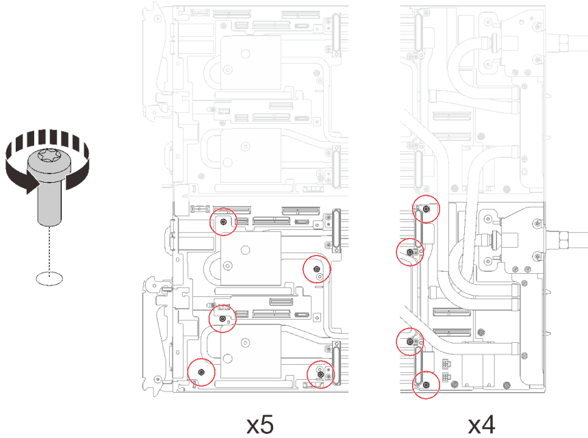
그림 190. 워터 루프 나사 제거
