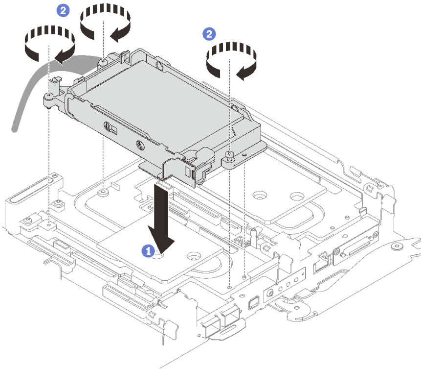
그림 80. 15mm 드라이브 케이지 어셈블리 1개 설치
