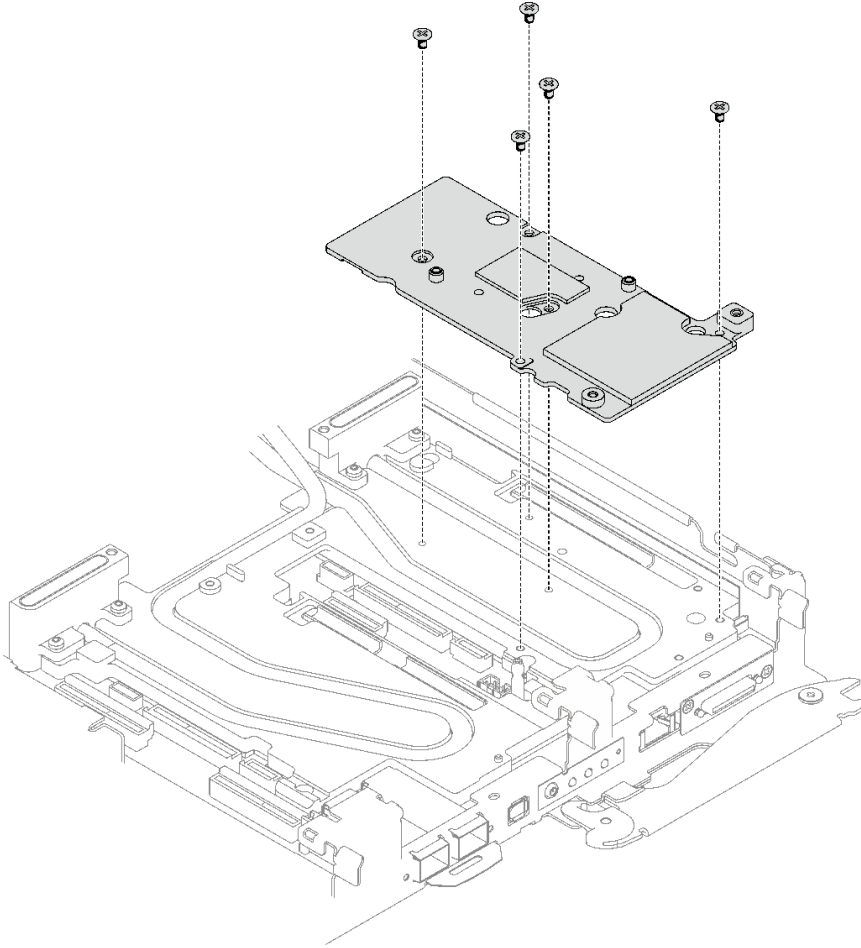
그림 172. 인터페이스판 설치
