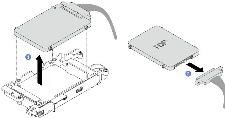
그림 65. 7mm 드라이브 제거
