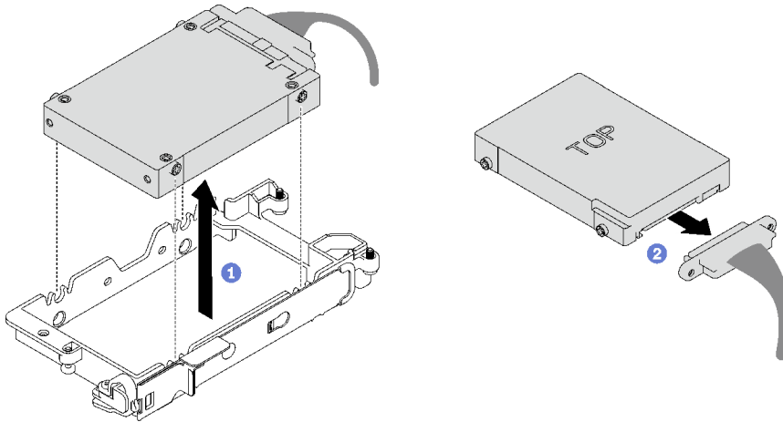
그림 66. 15mm 드라이브 제거
