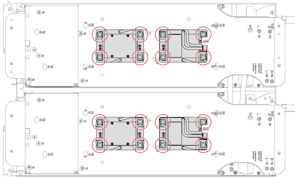
그림 46. Torx T30 고정 나사 고정하기
