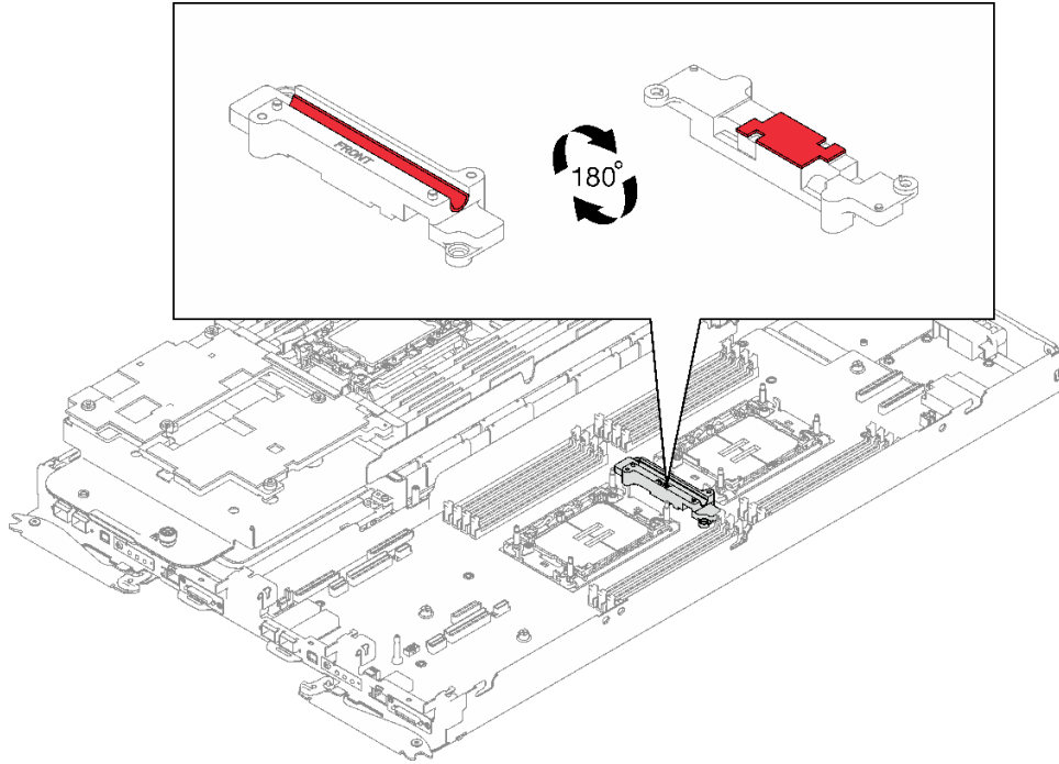
그림 239. VR 워터 루프 홈 갭 패드
