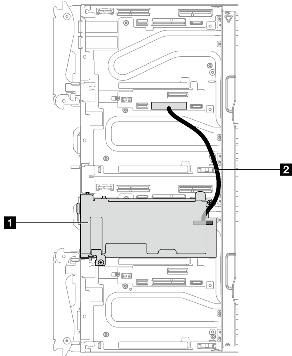
그림 242. ConnectX-7 NDR 200/ConnectX-7 NDR 400에 대한 공유 I/O 구성
