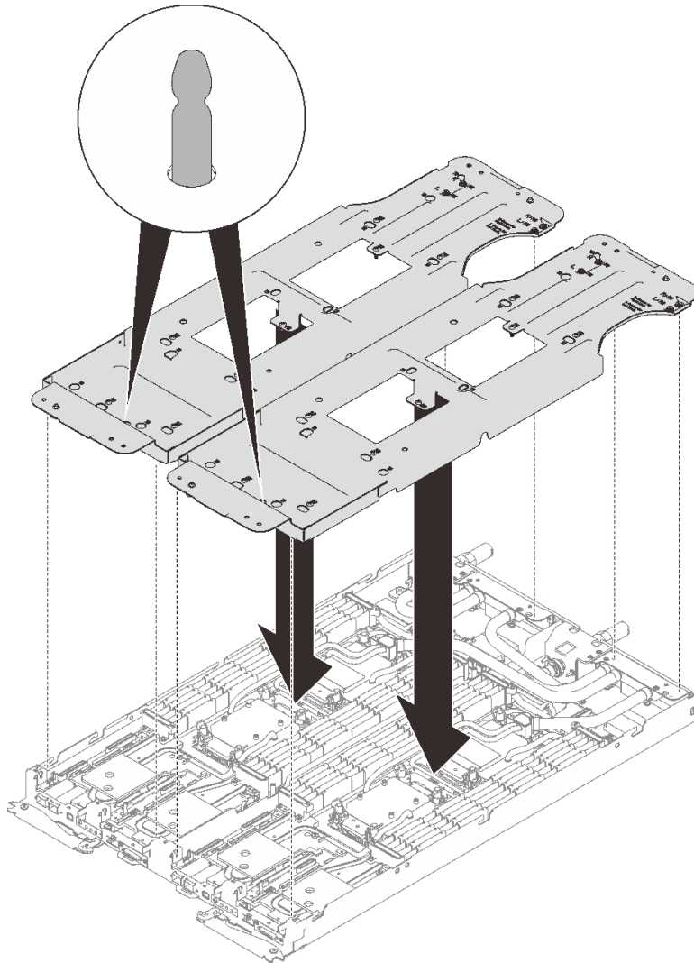
그림 25. 워터 루프 캐리어 설치
