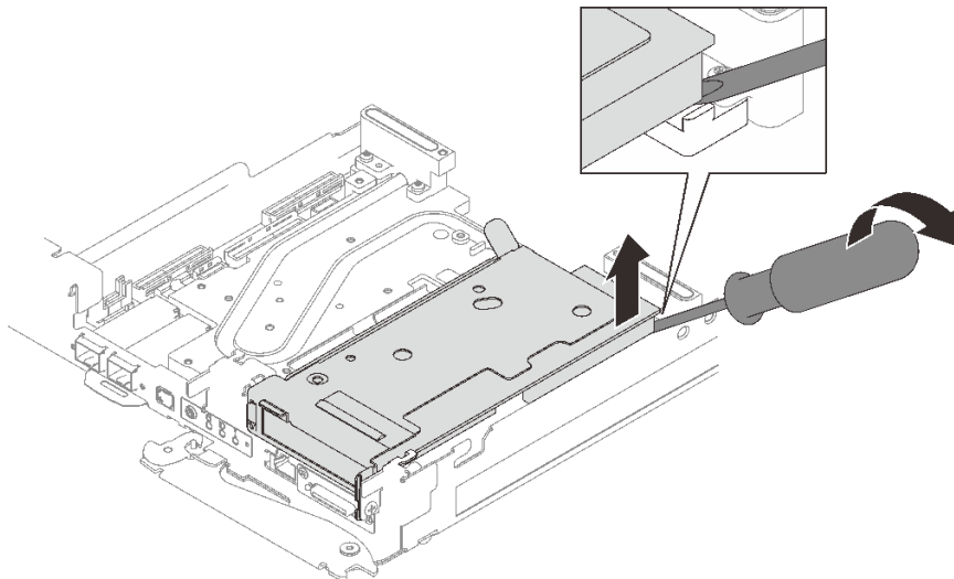
그림 177. 워터 루프 냉각판에서 PCIe 라이저 케이스 분리
