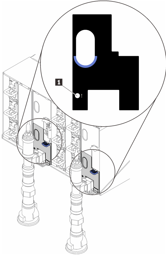
그림 256. 드립 센서 LED
