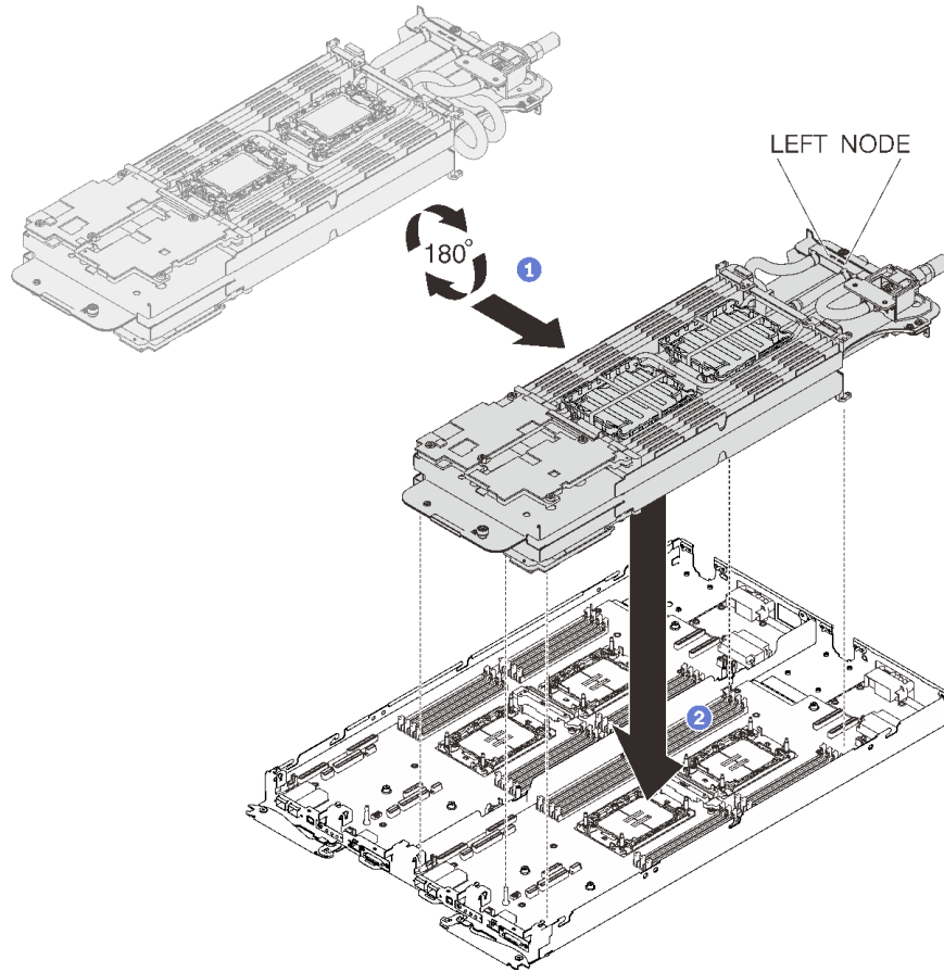
그림 43. 워터 루프 캐리어 설치
