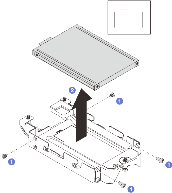
그림 105. 하단 E3.S 드라이브 제거
