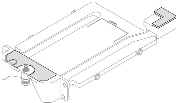
그림 110. 전도판 퍼티 패드 교체
