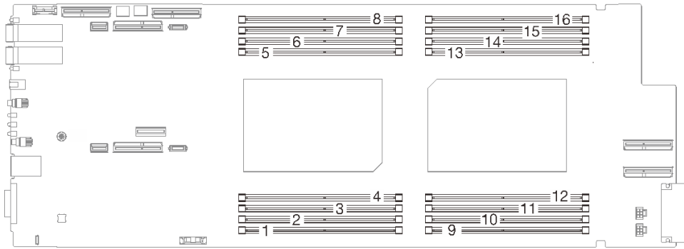
그림 139. 메모리 모듈 커넥터 위치
