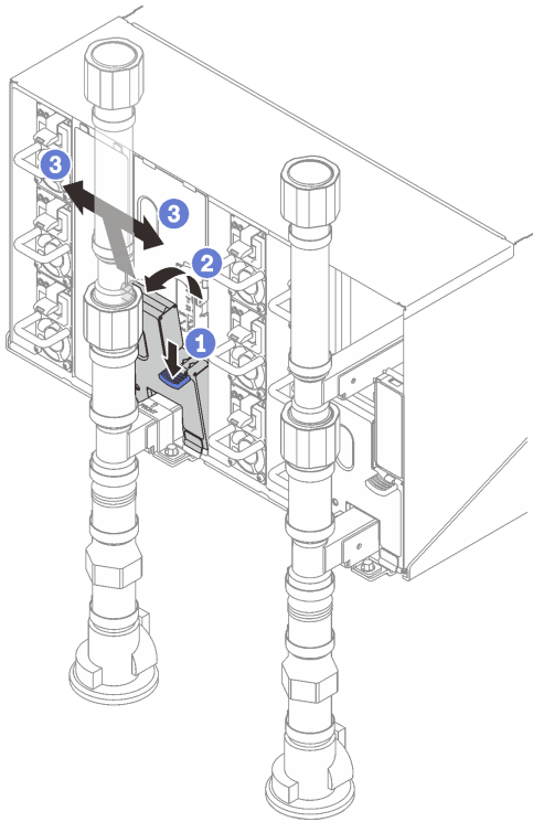
그림 259. 하단 EMC 실드 제거
