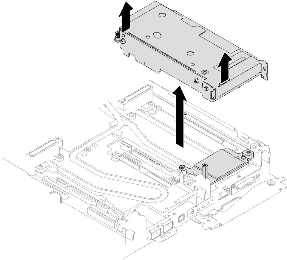
그림 153. PCIe 라이저 어셈블리 제거
