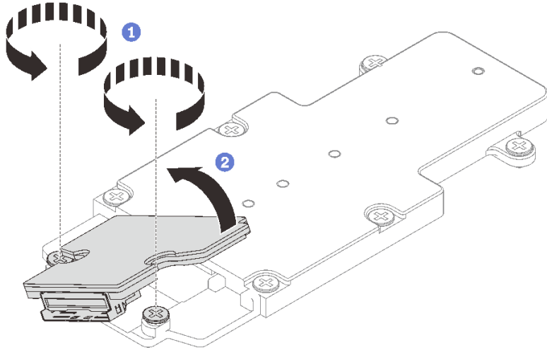
그림 126. M.2 백플레인 어셈블리 분해
