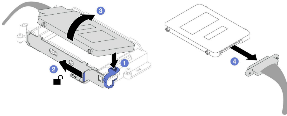
그림 87. 상단 드라이브 제거(7mm NVMe)
