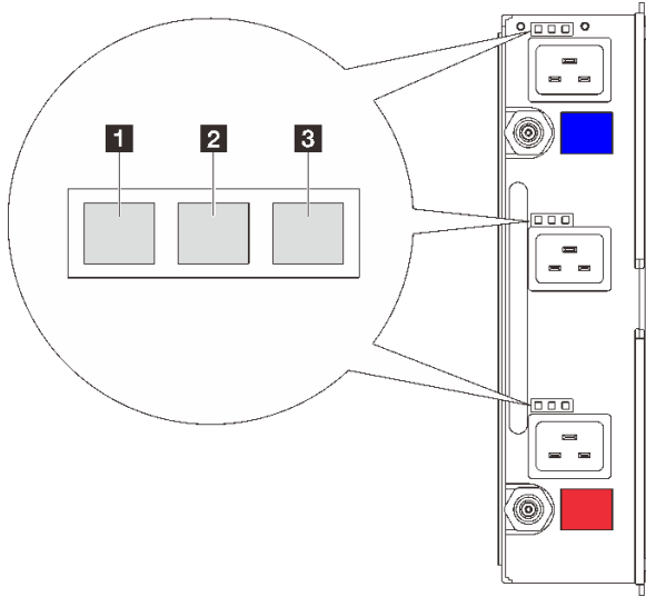
그림 255. DWC 전원 공급 장치 LED
