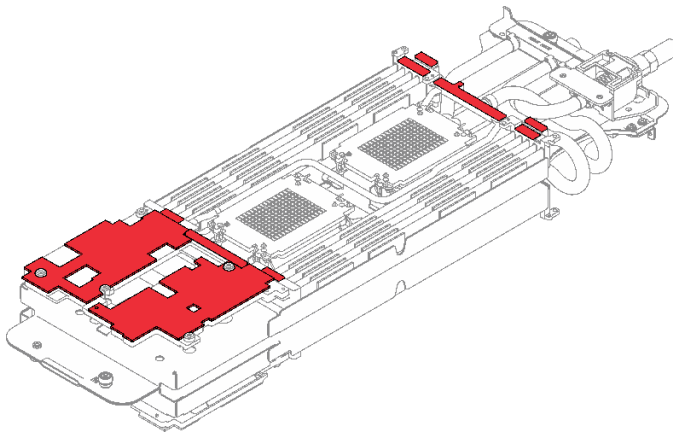
그림 198. 워터 루프 갭 패드
