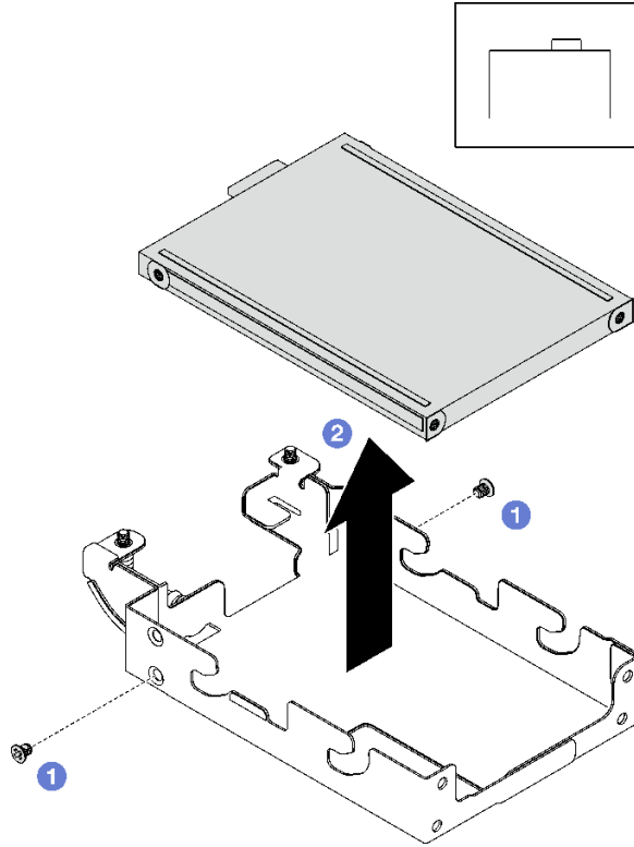
그림 107. 상단 E3.S 드라이브 제거
