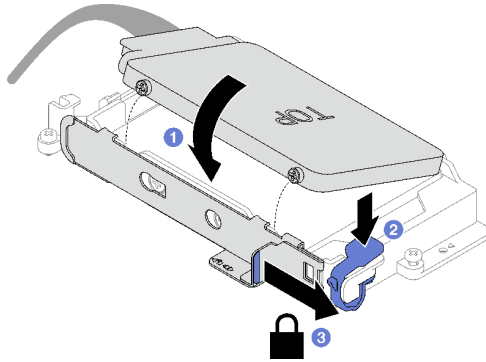
그림 74. 위쪽 드라이브 설치
