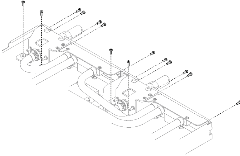
그림 23. 킥 커넥트 나사 제거
