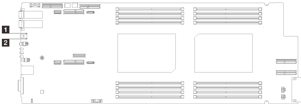
그림 257. 시스템 보드 LED
