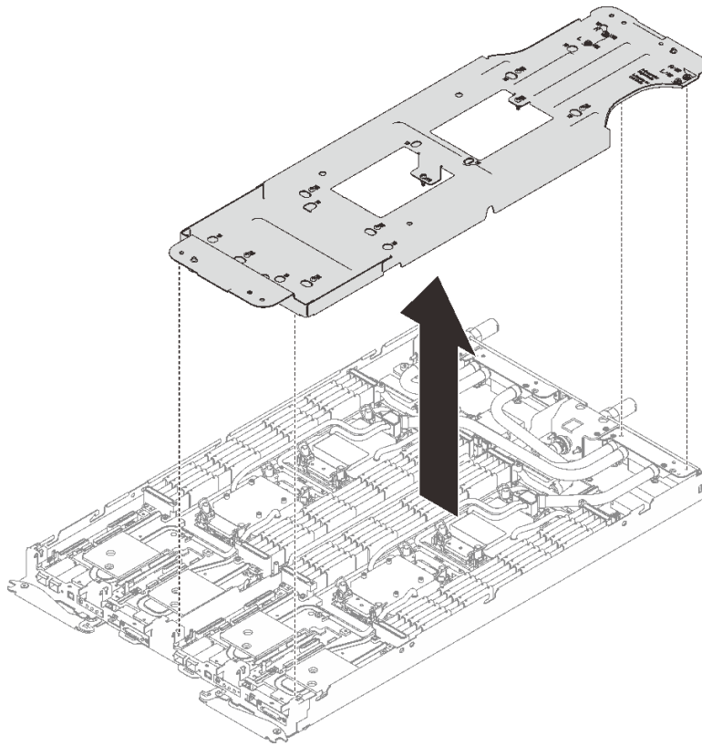
그림 202. 워터 루프 캐리어 제거
