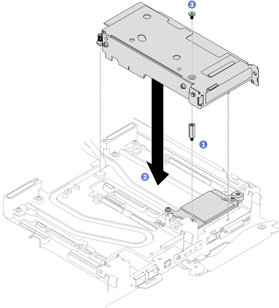
그림 160. PCIe 라이저 어셈블리 설치
