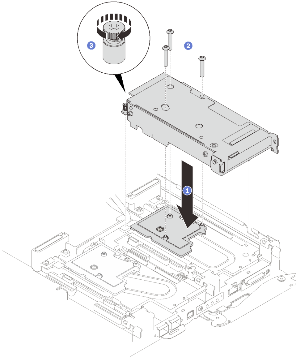
그림 188. PCIe 라이저 어셈블리 설치
