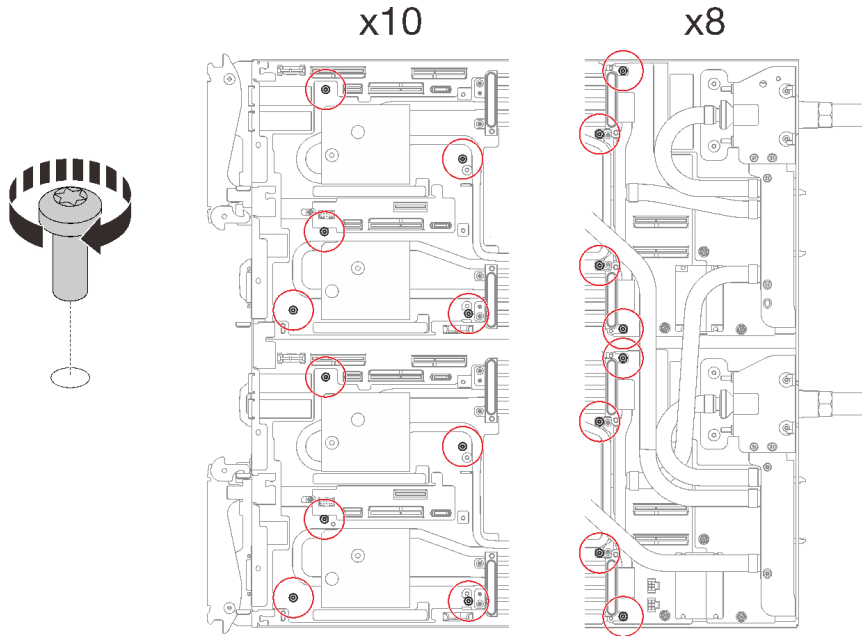
그림 49. 워터 루프 나사 설치
