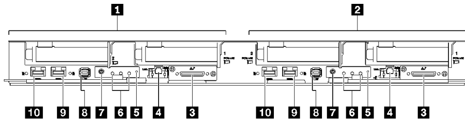
그림 2. SD650 V3 트레이
