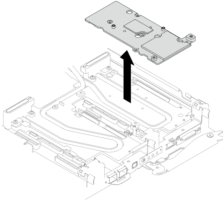
그림 168. 인터페이스판 제거
