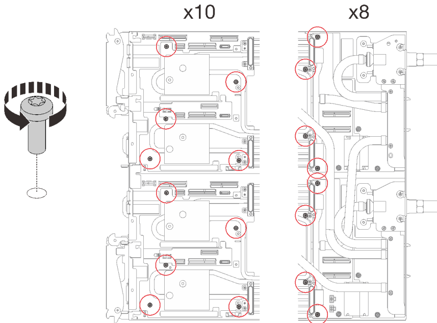
그림 24. 워터 루프 나사 제거
