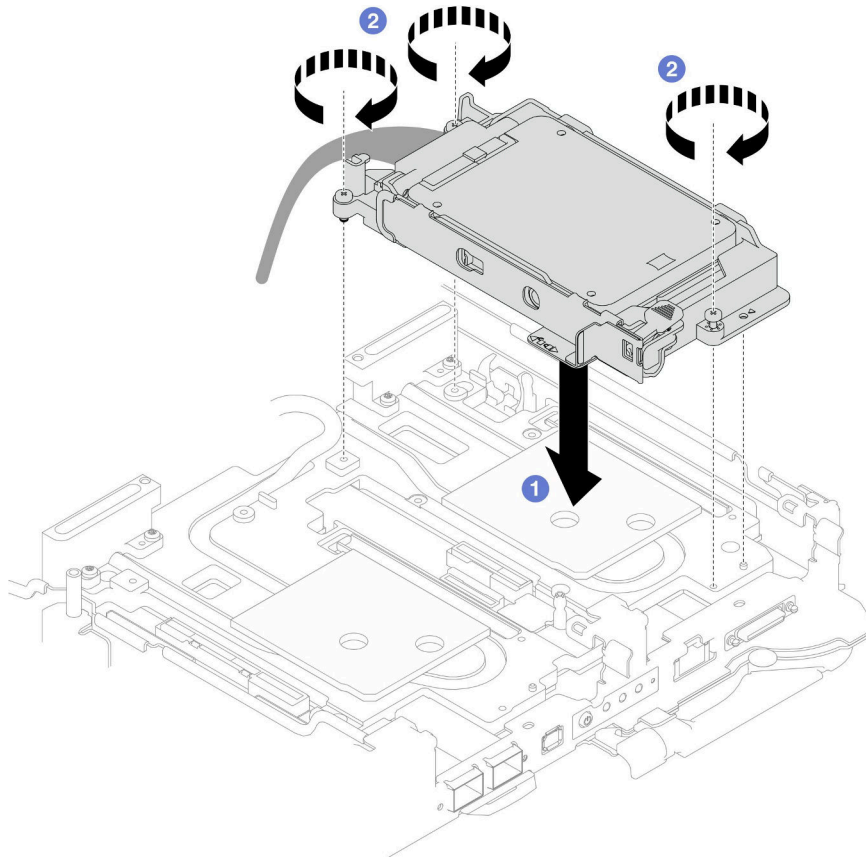
그림 97. 7mm NVMe 드라이브 케이징 어셈블리 설치
