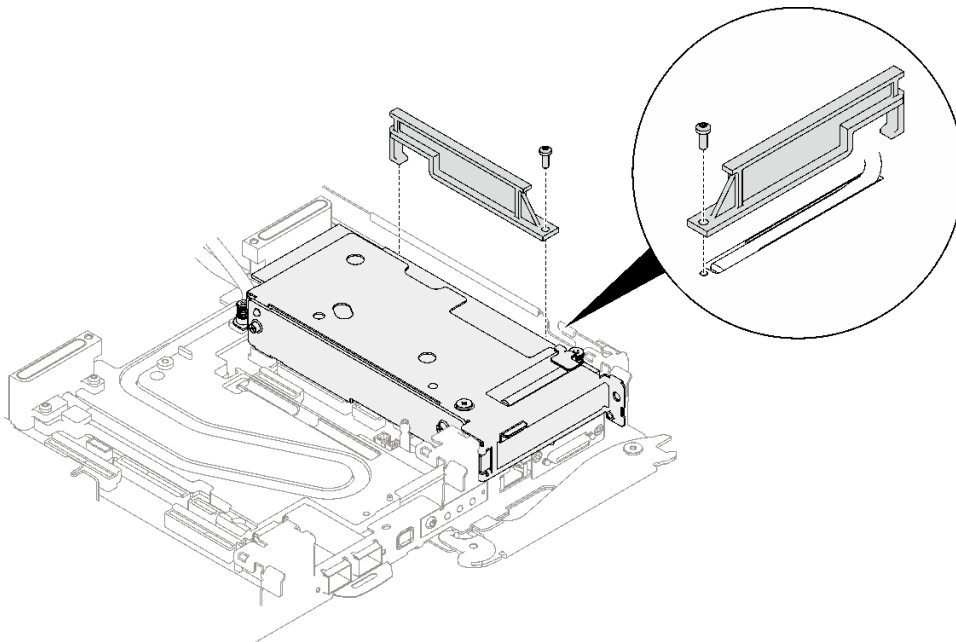
그림 162. 히트파이프 빔 설치
