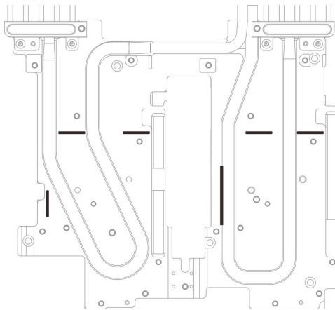
그림 94. 갭 패드를 맞추기 위한 워터 루프의 표시
