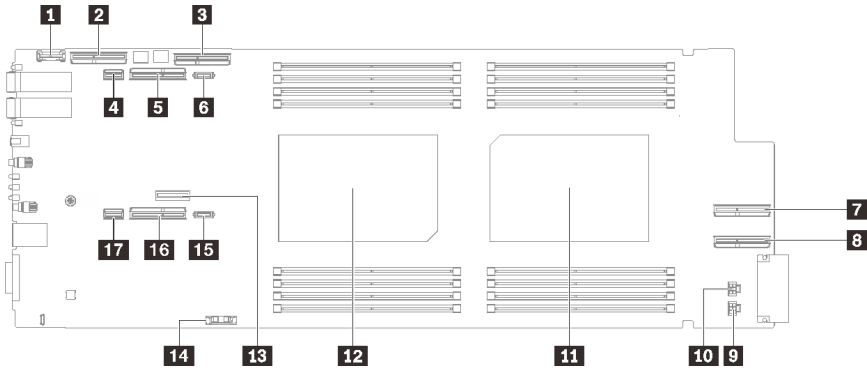
그림 5. 컴퓨팅 노드 시스템 보드의 내부 커넥터
