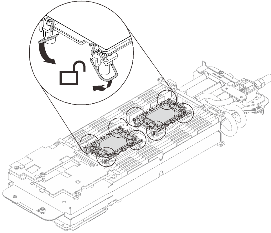
그림 41. 프로세서 잠금 해제 위치
