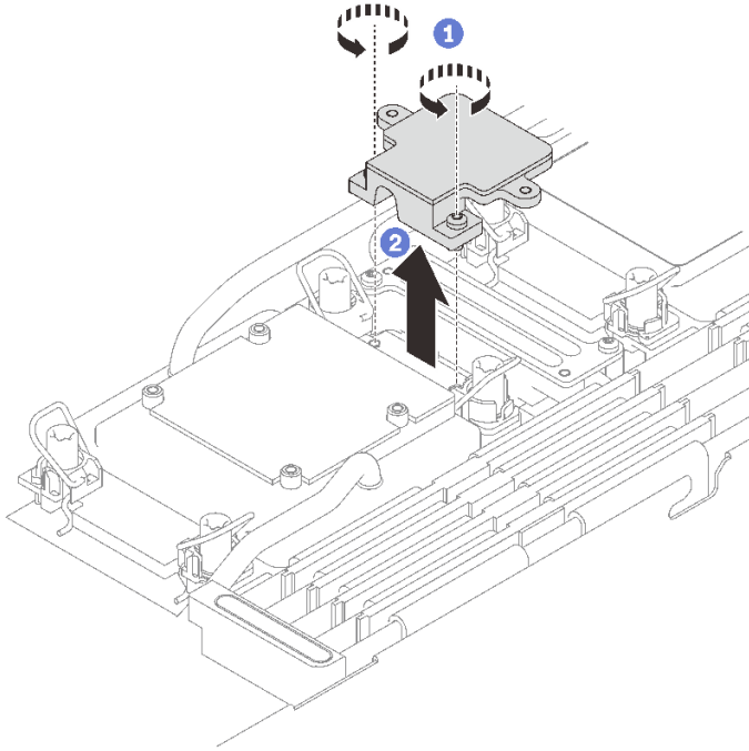
그림 125. M.2 백플레인 냉각판 제거
