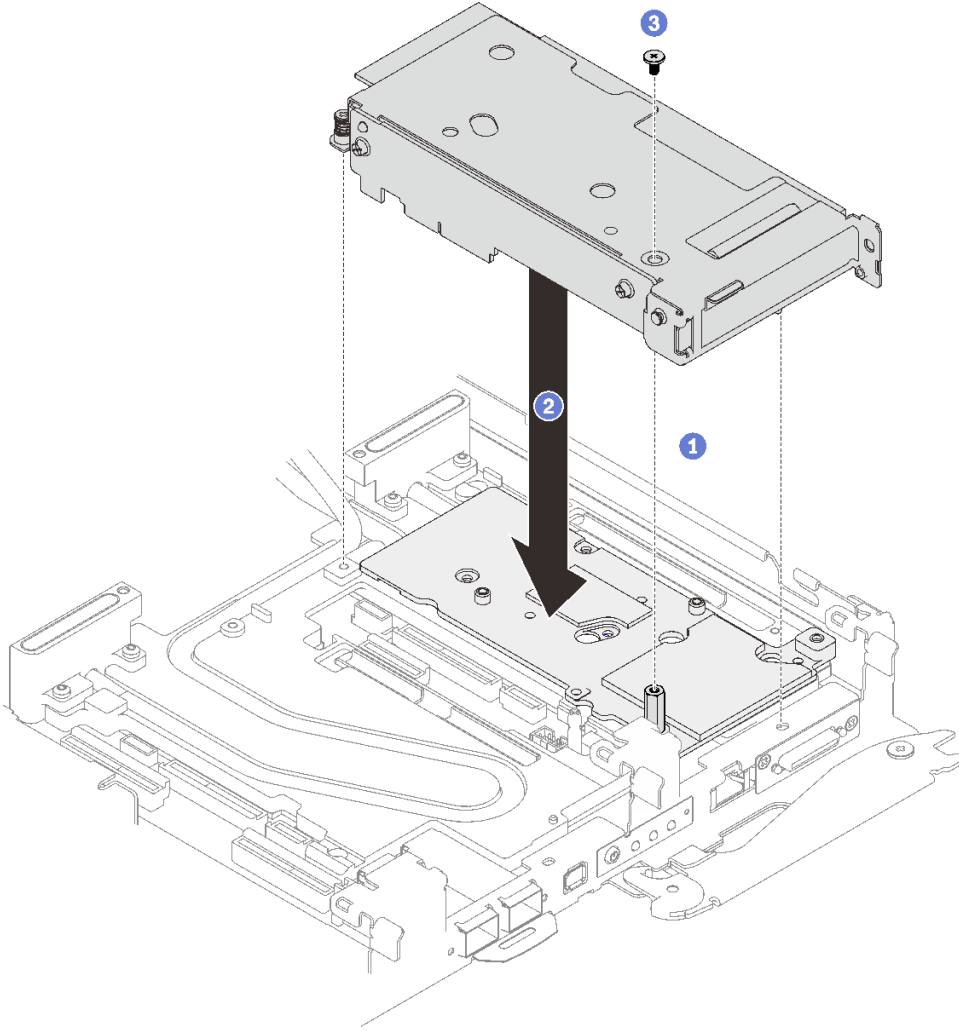
그림 174. PCIe 라이저 어셈블리 설치
