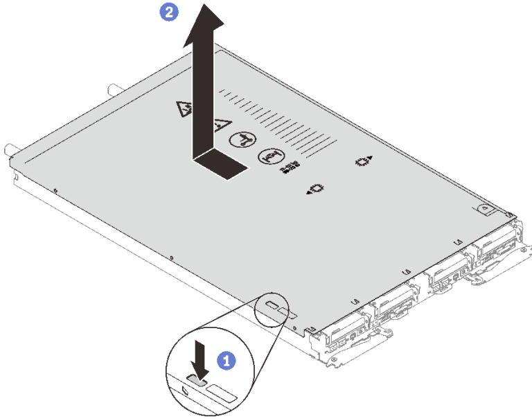
그림 18. 트레이 덮개 제거
