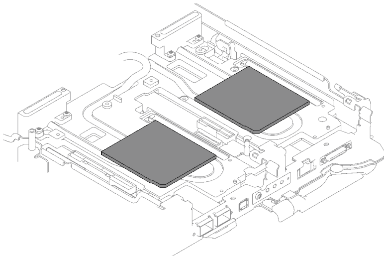
그림 96. 갭 패드 위치
