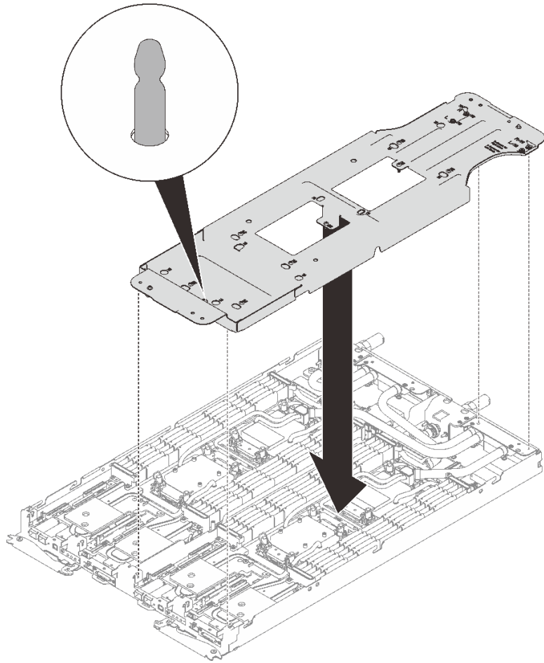
그림 210. 워터 루프 캐리어 설치
