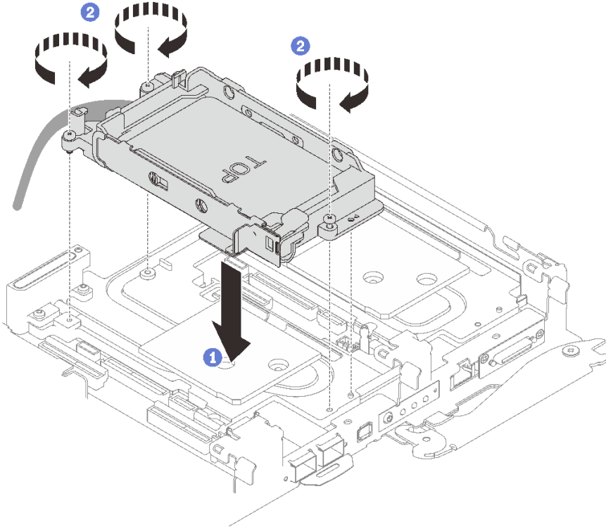
그림 81. 7mm 드라이브 케이지 어셈블리 1개 설치
