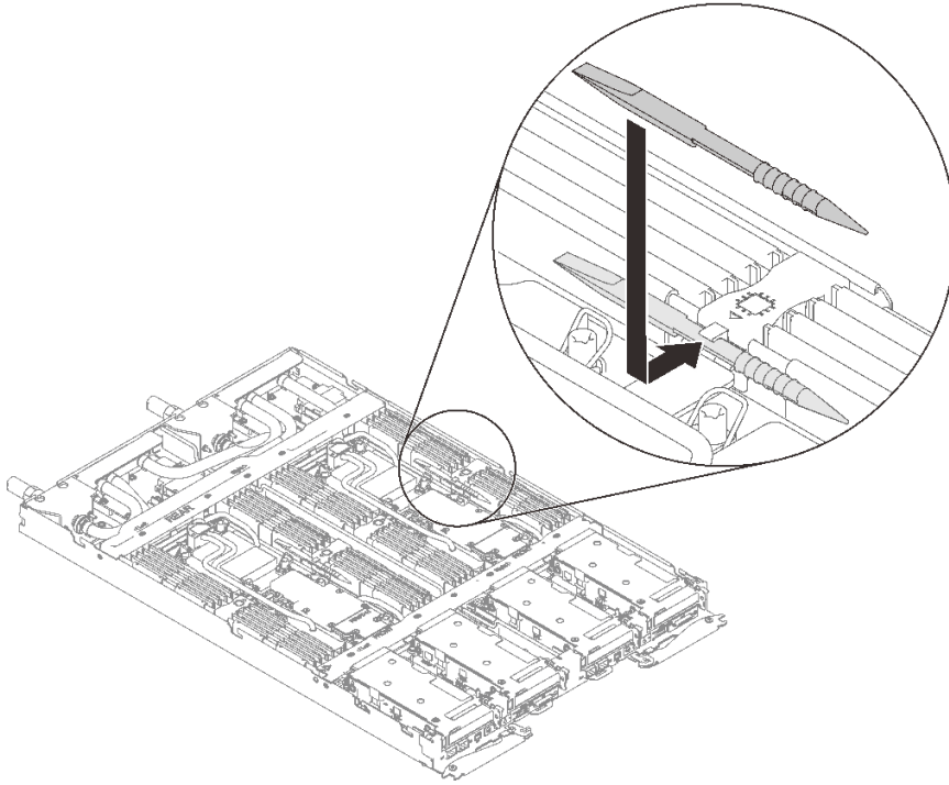
그림 138. 메모리 모듈 도구 설치
