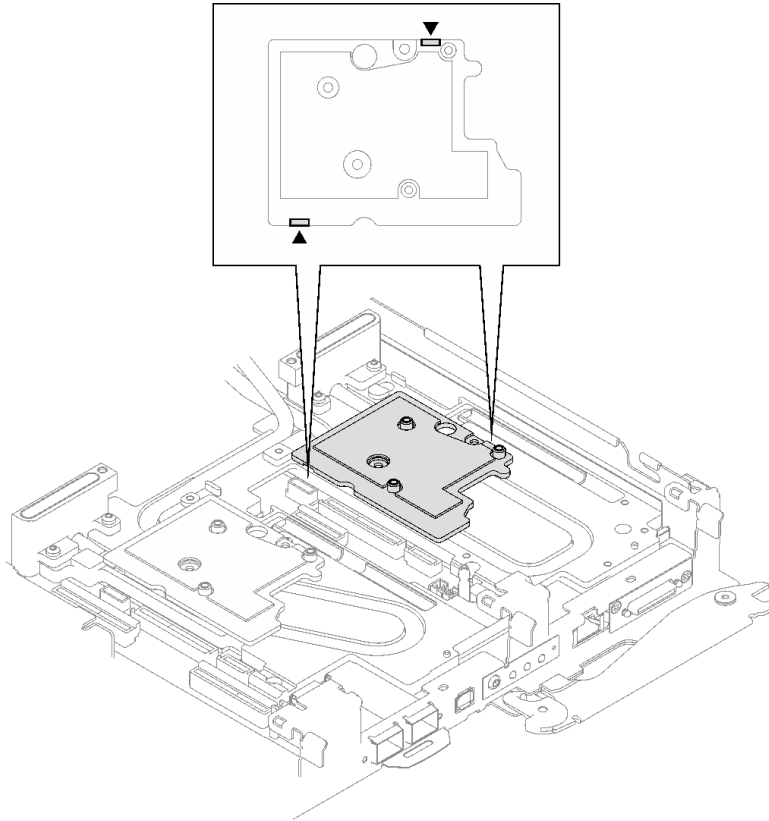
그림 180. 인터페이스판 하단의 구멍 위치
