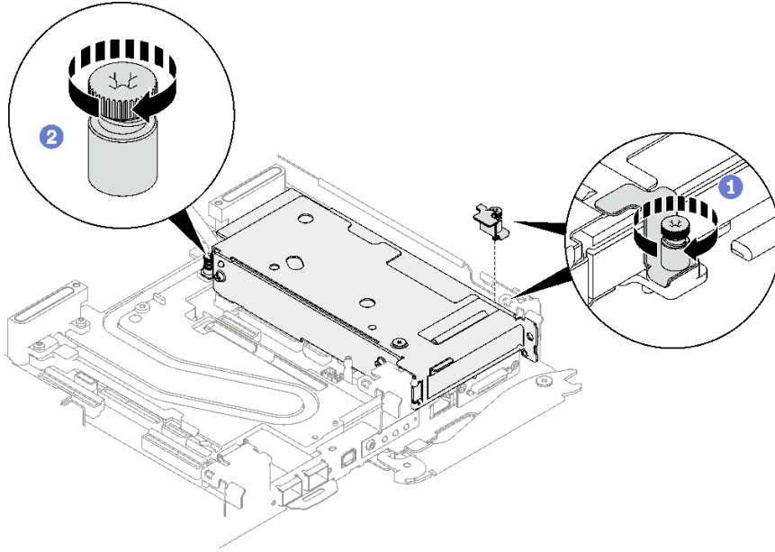
그림 161. 클램프 브래킷 고정 나사 설치
