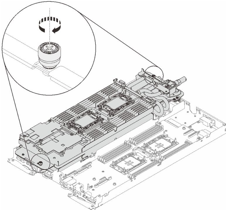
그림 29. 고정 나비 나사 조이기
