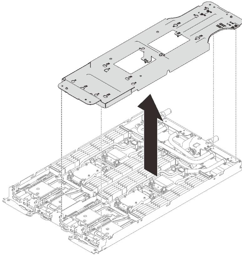
그림 229. 워터 루프 캐리어 제거
