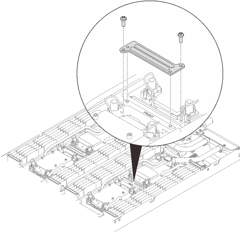
그림 232. VR 클램프판 설치
