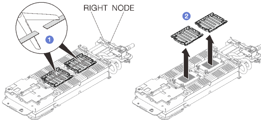
그림 222. 플라스틱 그리스 덮개 제거
