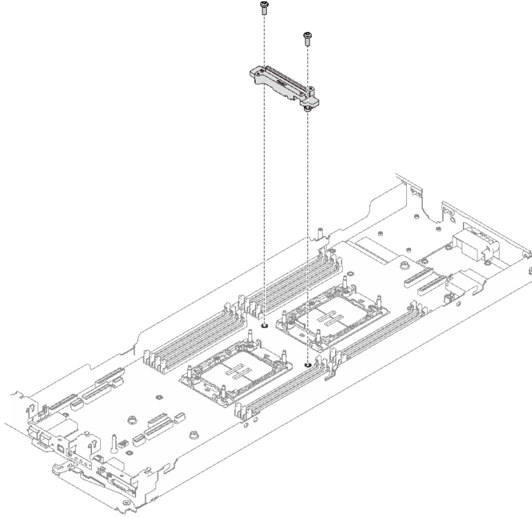
그림 240. VR 워터 루프 홀 설치
