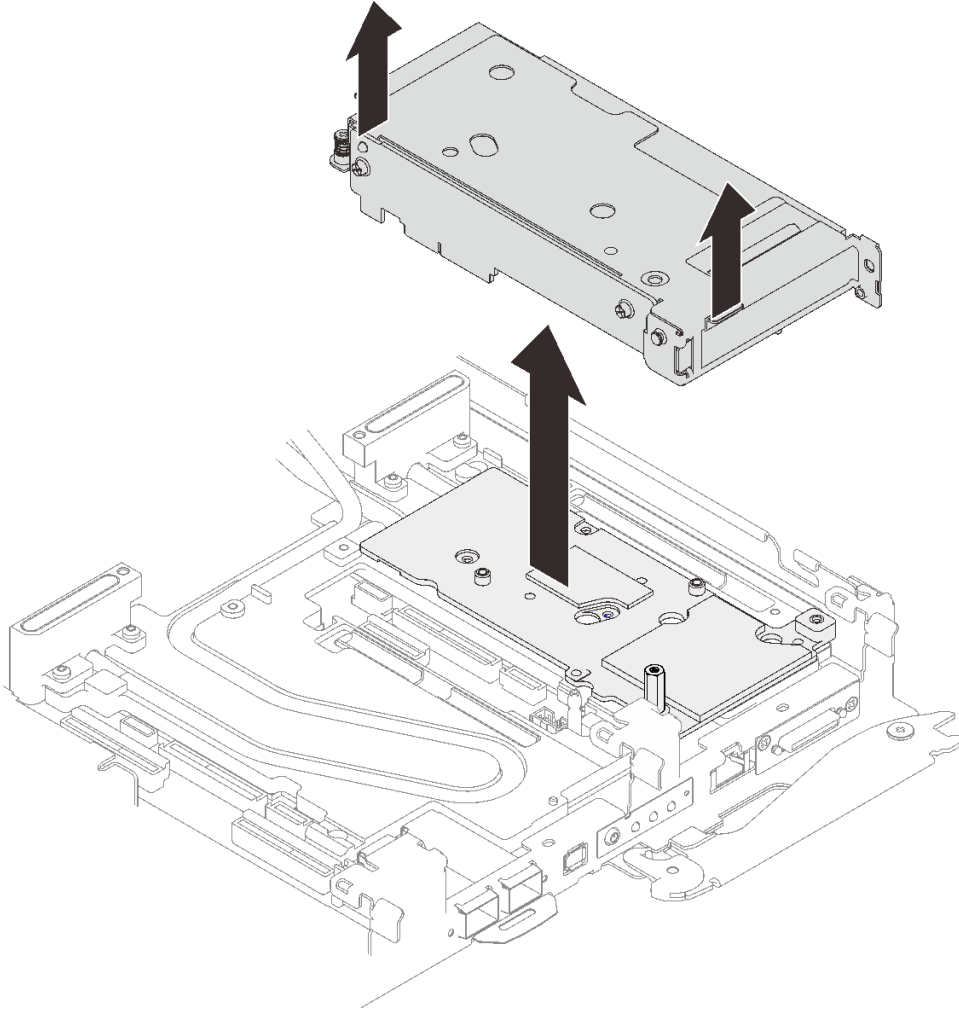
그림 164. PCIe 라이저 어셈블리 제거
