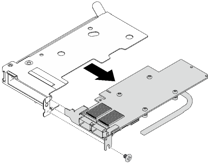
그림 145. PCIe 어댑터 제거
