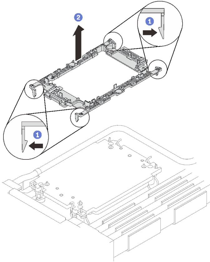
그림 32. 프로세서 고정장치 제거
