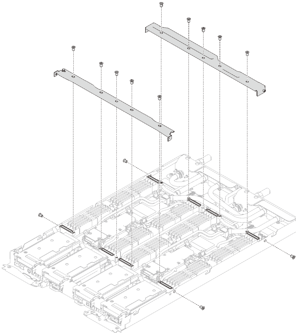
그림 20. 십자형 브레이스 제거(SD650 V3)
