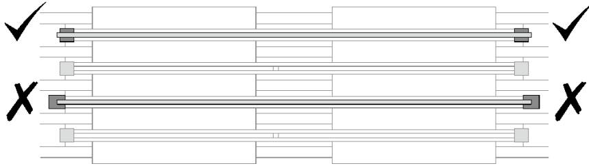
그림 143. 메모리 모듈 커넥터의 해제 및 잠긴 고정 클립
