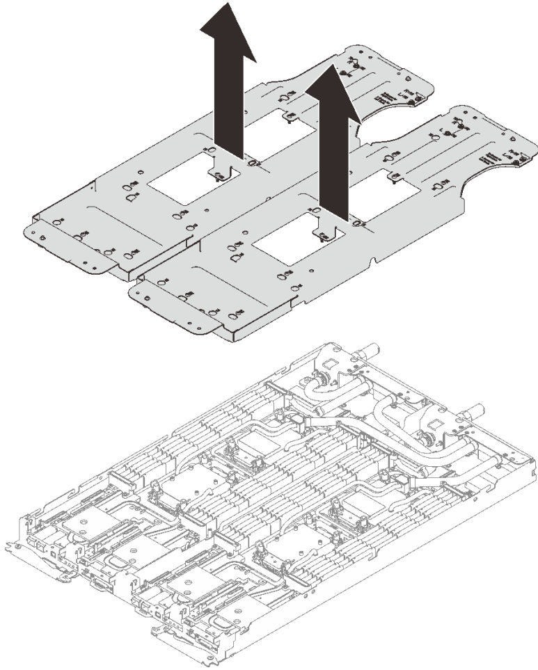
그림 48. 워터 루프 캐리어 제거
