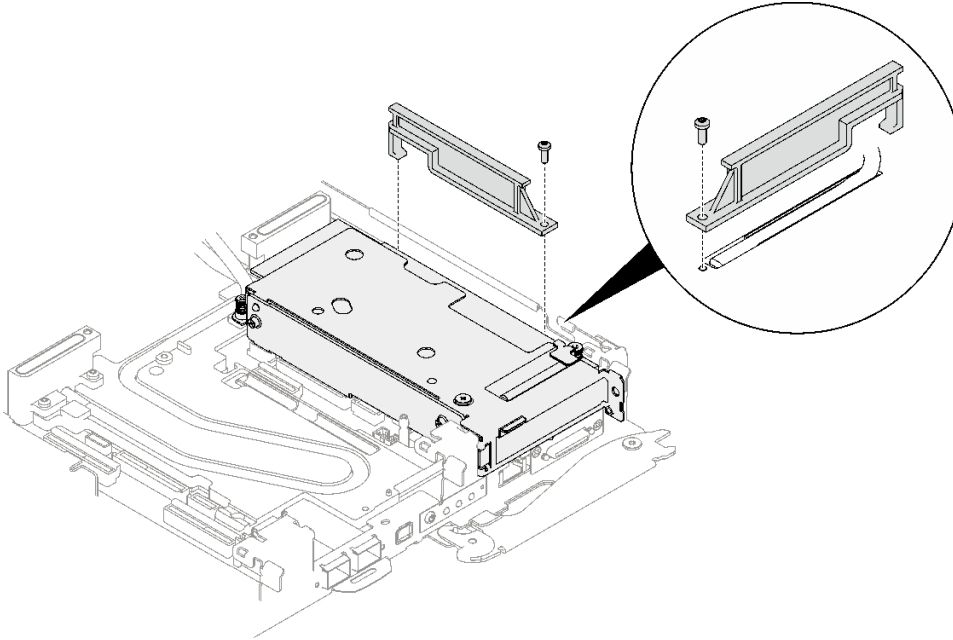
그림 151. 히트파이프 빔 제거
