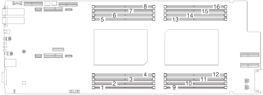
그림 14. 메모리 모듈 및 프로세서 레이아웃
