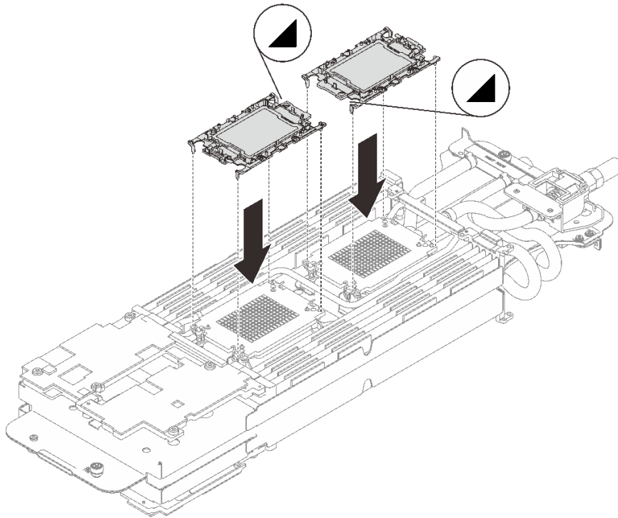
그림 223. 프로세서 설치
