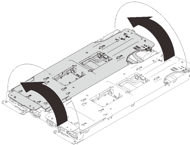
그림 45. 워터 루프 펼치기
