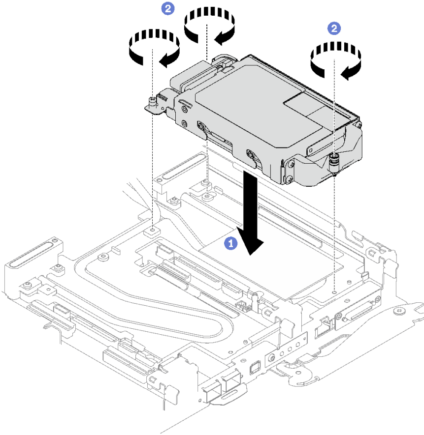
그림 119. E3.S 드라이브 케이징 어셈블리 설치
