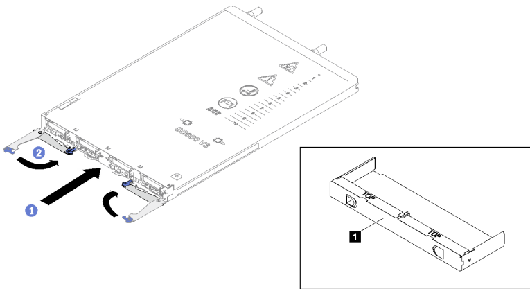
그림 17. 트레이 설치
