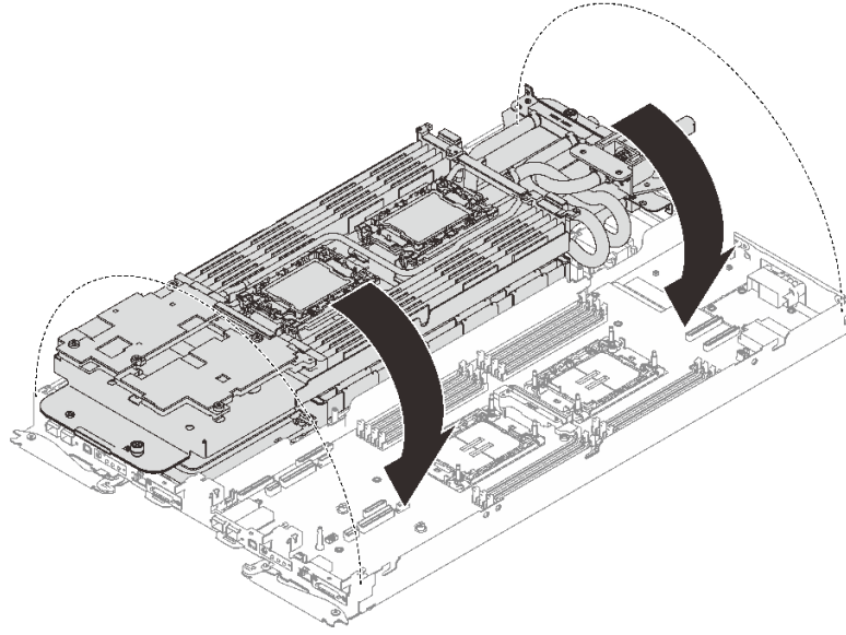
그림 226. 워터 루프 설치
