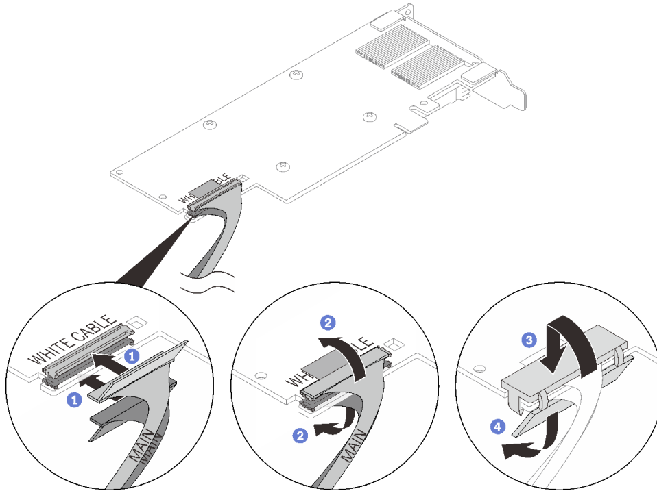
그림 149. PCIe 어댑터 케이블 설치
