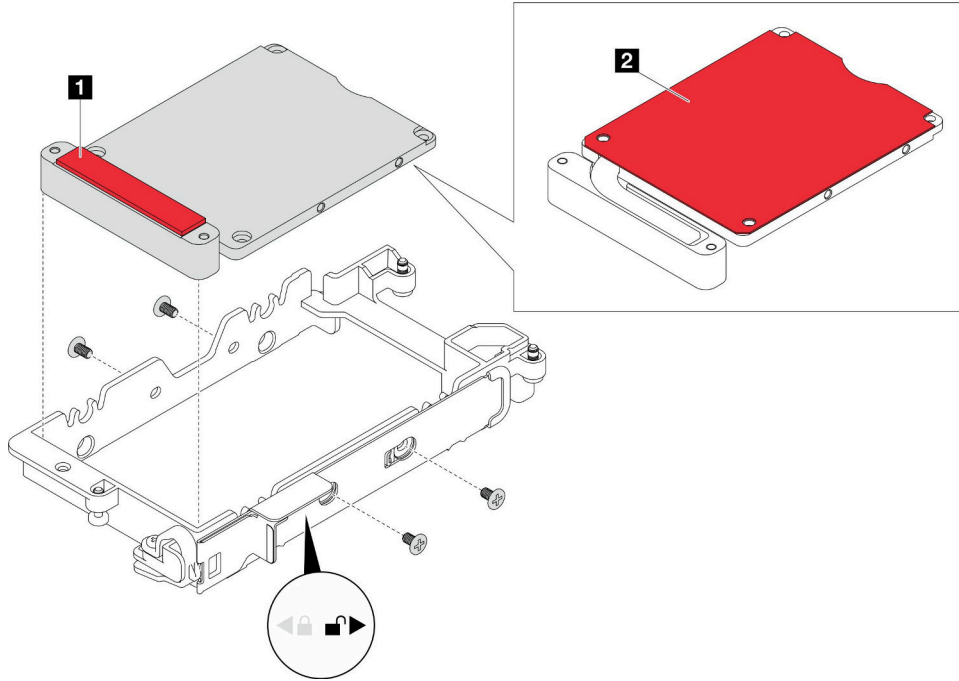
그림 72. 전도판 설치
