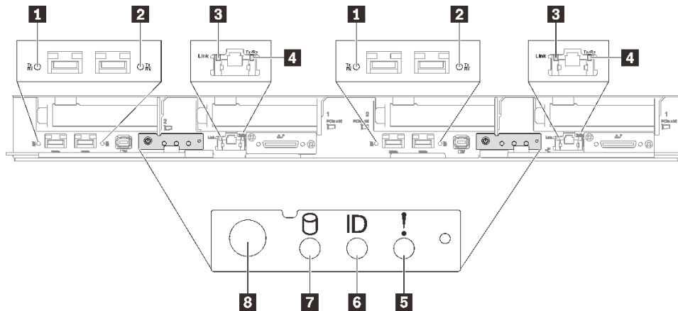
그림 252. SD650 V3 트레이 앞면 LED
