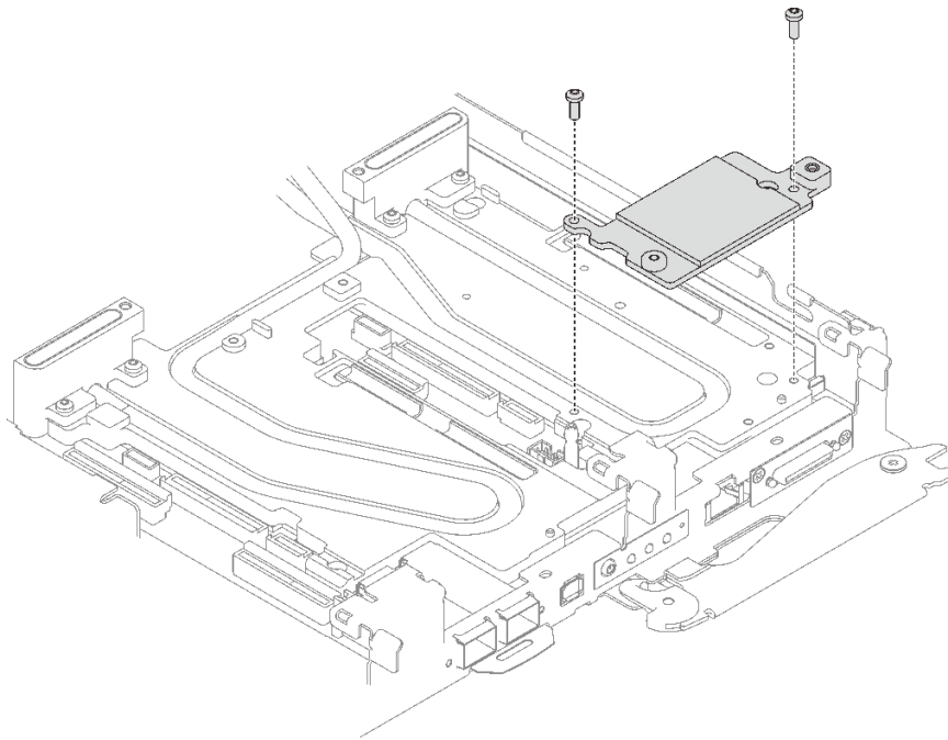
그림 158. 인터페이스판 설치
