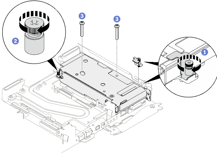
그림 175. 클램프 브래킷 고정 나사 설치
