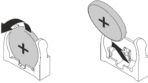
그림 53. CMOS 배터리 제거
