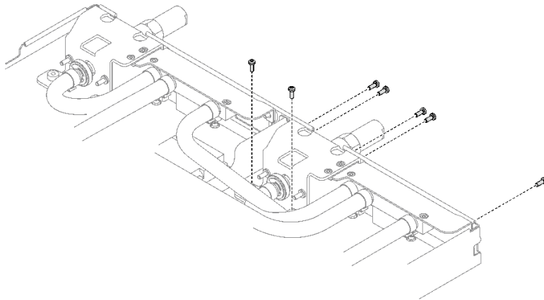
그림 231. 퀵 커넥트 나사 설치
