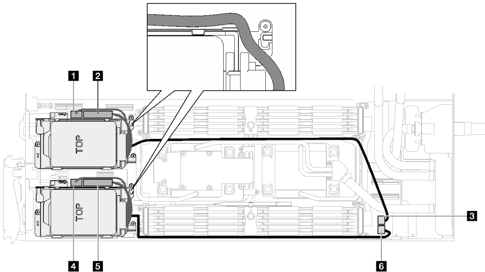
그림 84. 드라이브 어셈블리 케이블 배선
