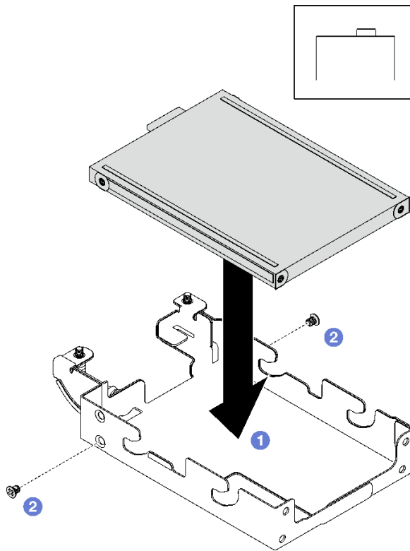
그림 108. 상단 E3.S 드라이브 설치
