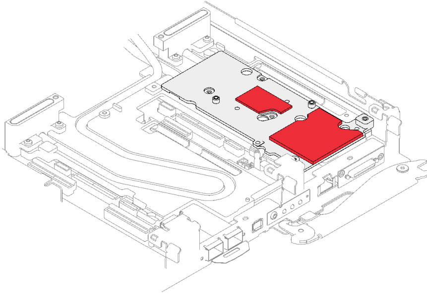
그림 173. CX-7 NDR 200용 냉각판의 인터페이스 패드
