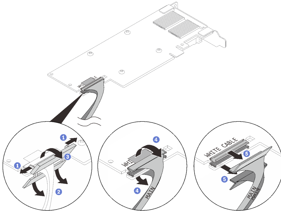
그림 146. PCIe 어댑터 케이블 제거
