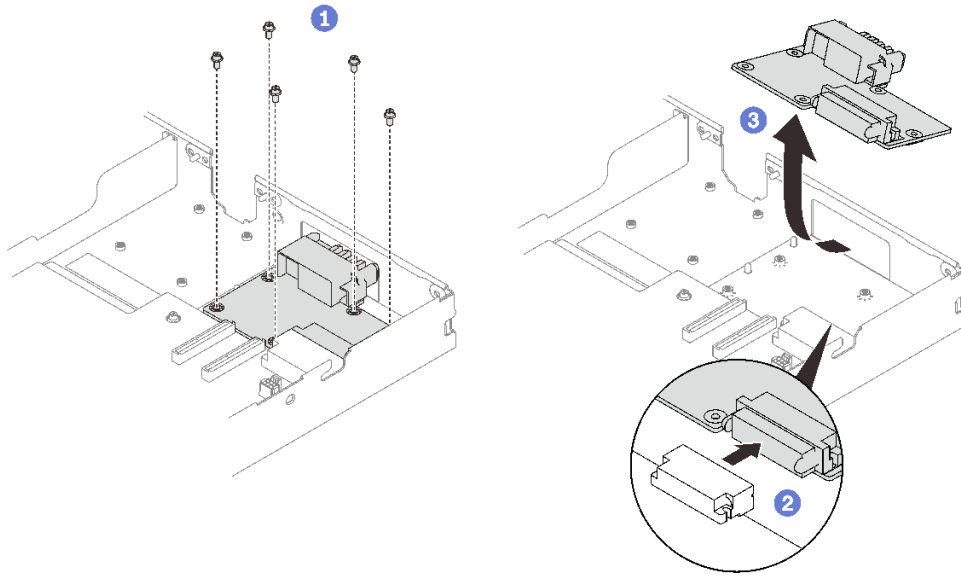
그림 196. 전원 분배 보드 제거
