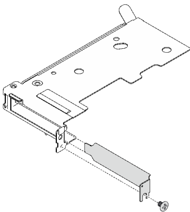
그림 147. 필러 설치
