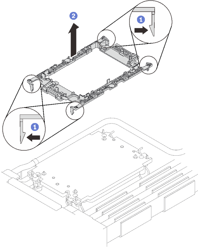
그림 216. 프로세서 고정장치 제거
