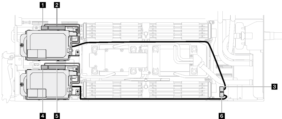
그림 99. E3.S 드라이브 케이블 배선
