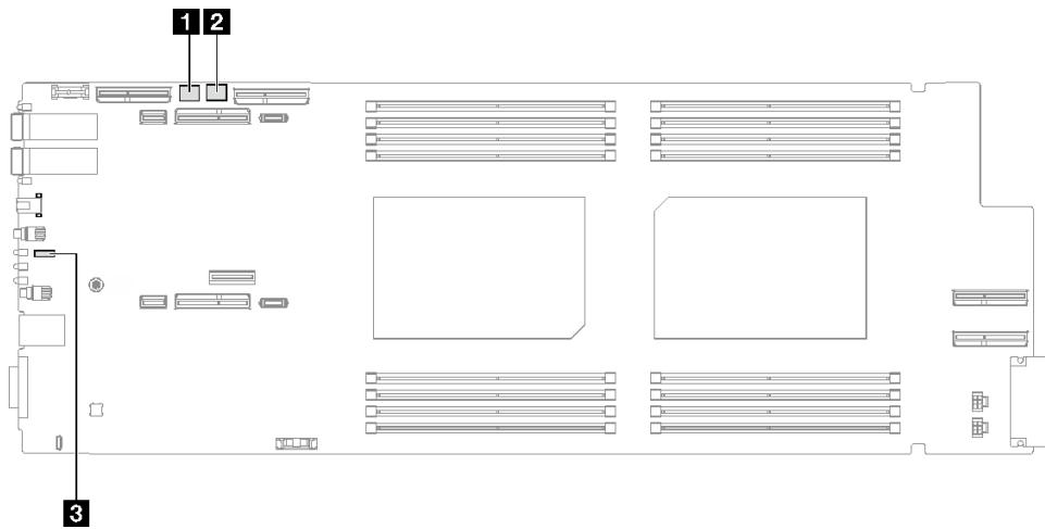
그림 7. 컴퓨팅 노드 시스템 보드의 스위치
