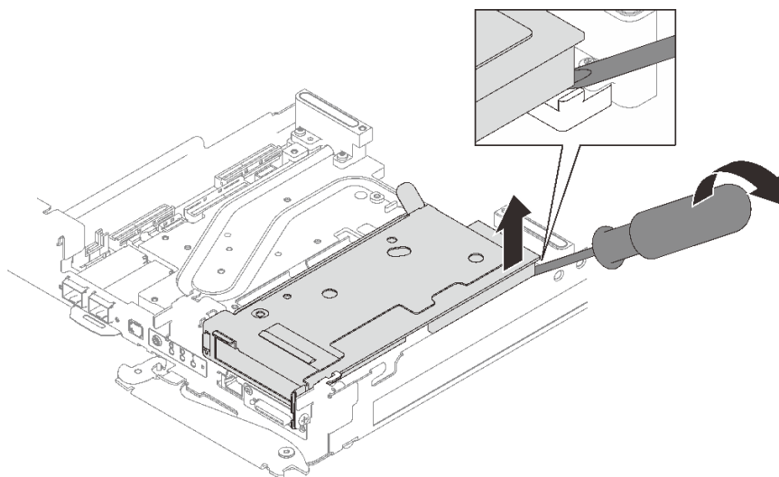
图 177. 将 PCIe 转接卡架从水循环模块冷却板上松开
