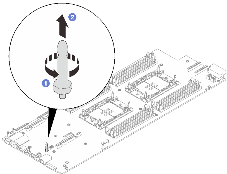
图 236. 卸下导销
