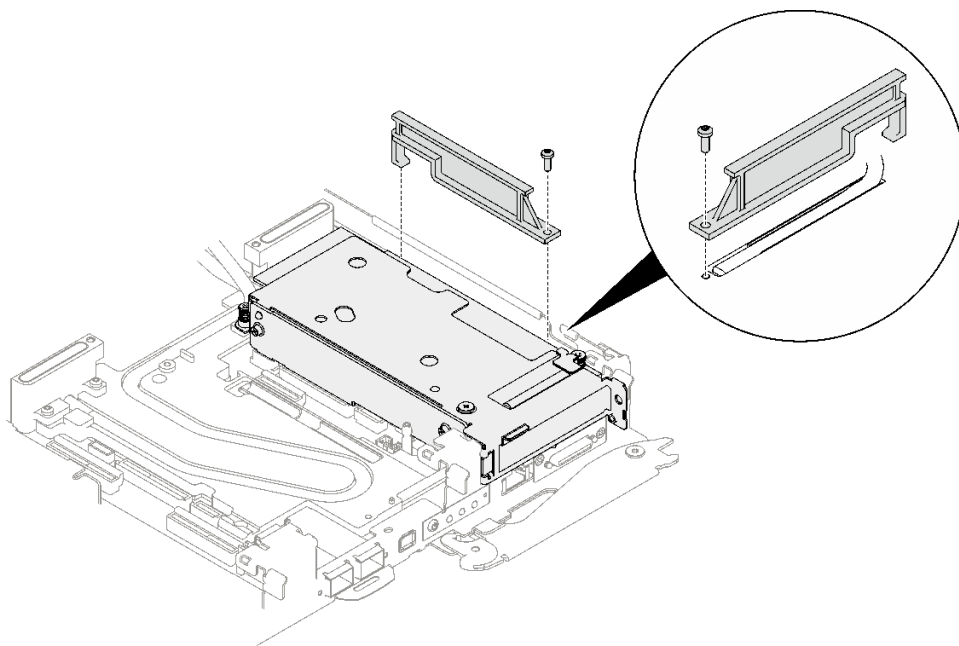
图 151. 卸下导热管架
