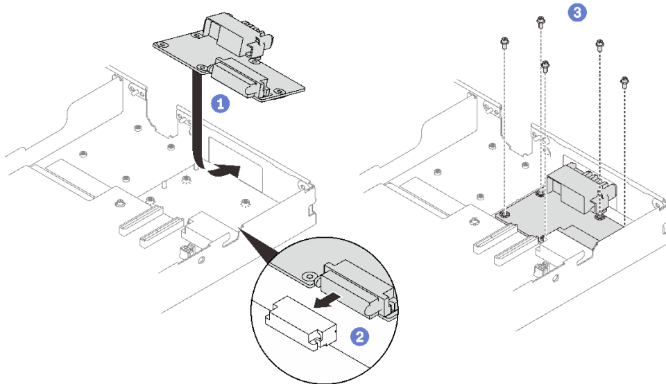
图 197. 安装配电板
