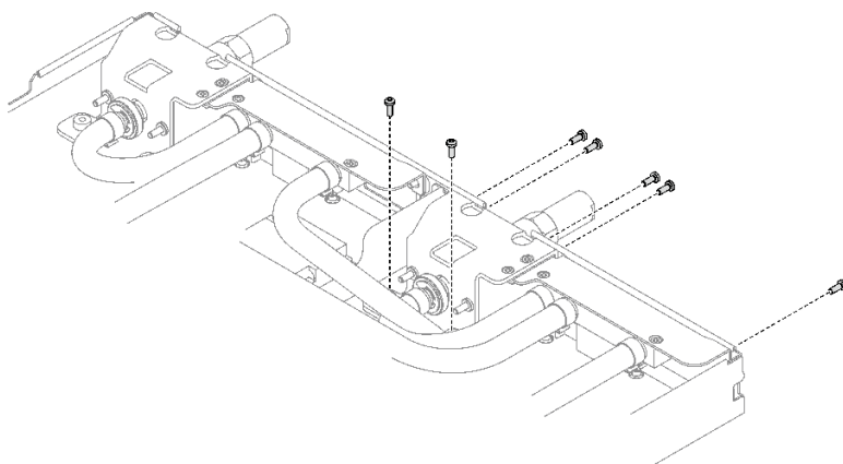
图 204. 安装快接件螺钉
