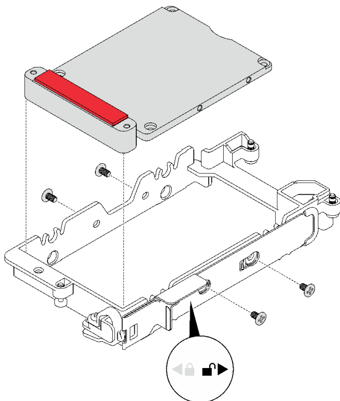
图 69. 卸下导电板
