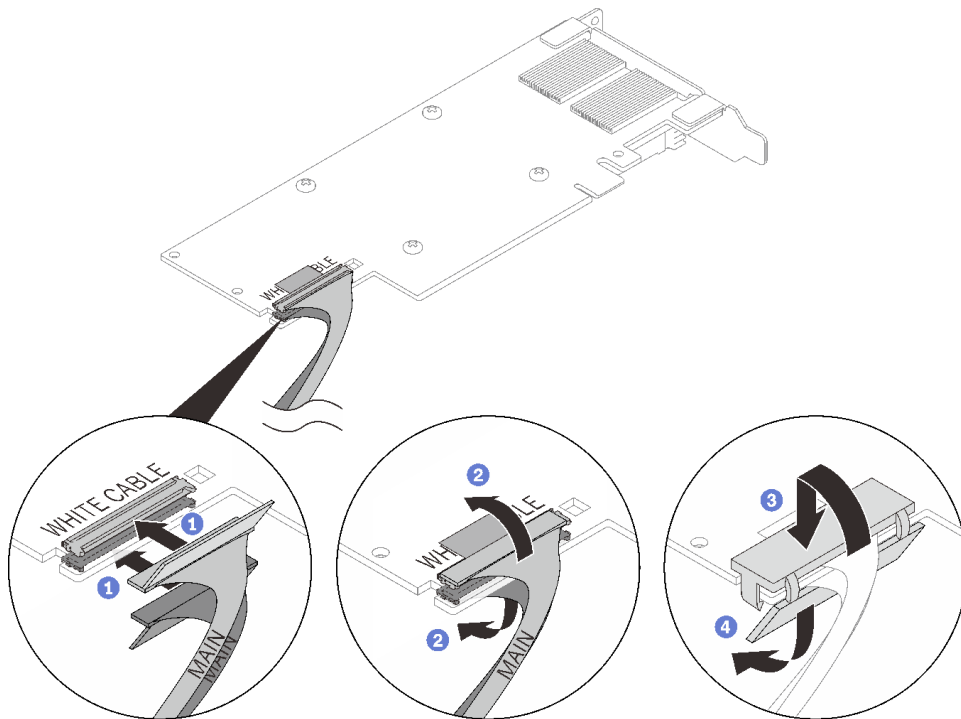
图 149. 安装 PCIe 适配器线缆
