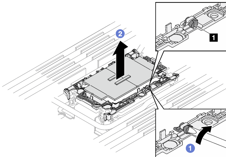
图 31. 卸下处理器 (Intel® Xeon® CPU Max 处理器)
