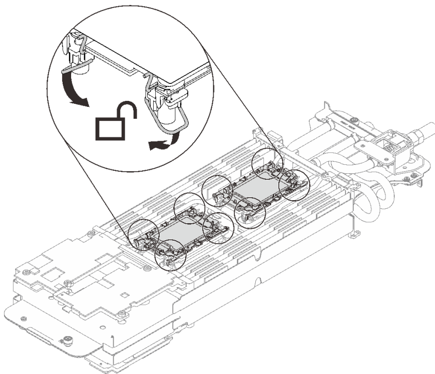
图 41. 处理器解锁位置
