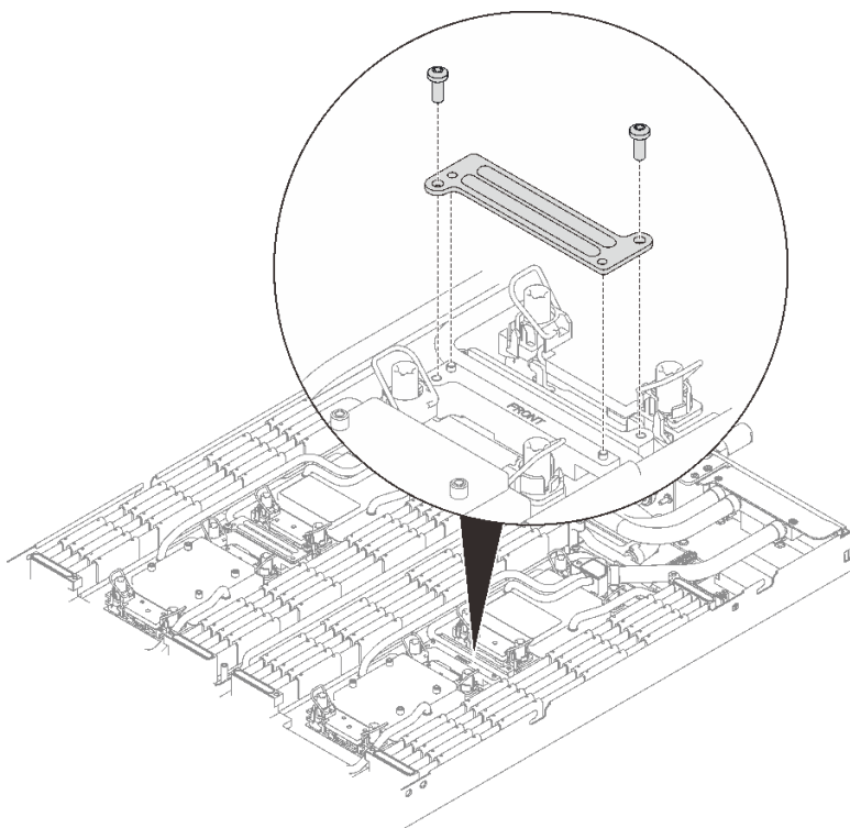
图 205. 安装 VR 夹板
