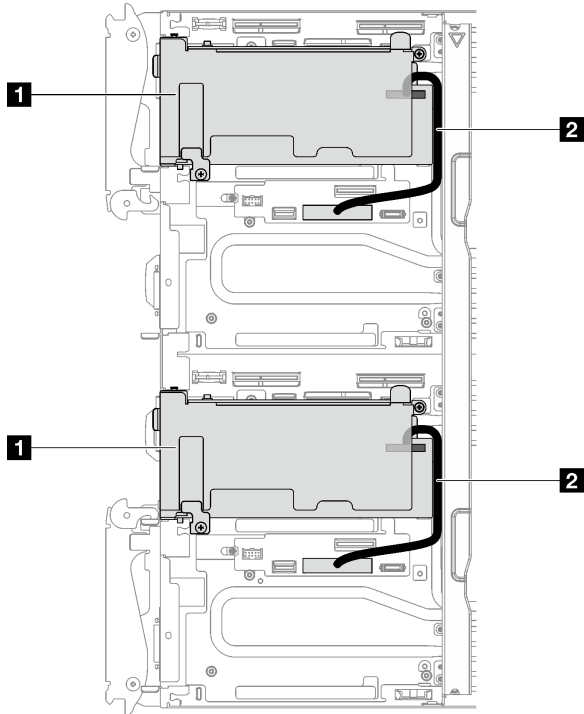
图 243. ConnectX-7 NDR 200/ConnectX-7 NDR 400 插槽直连配置的线缆布放
