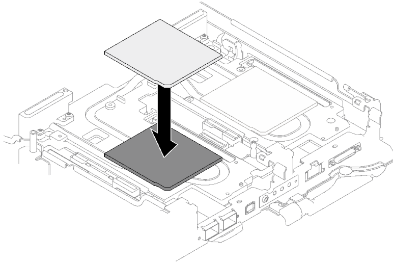
图 95. 更换间隙垫
