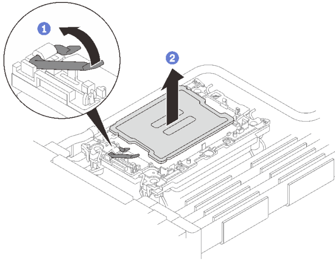
图 30. 卸下处理器
