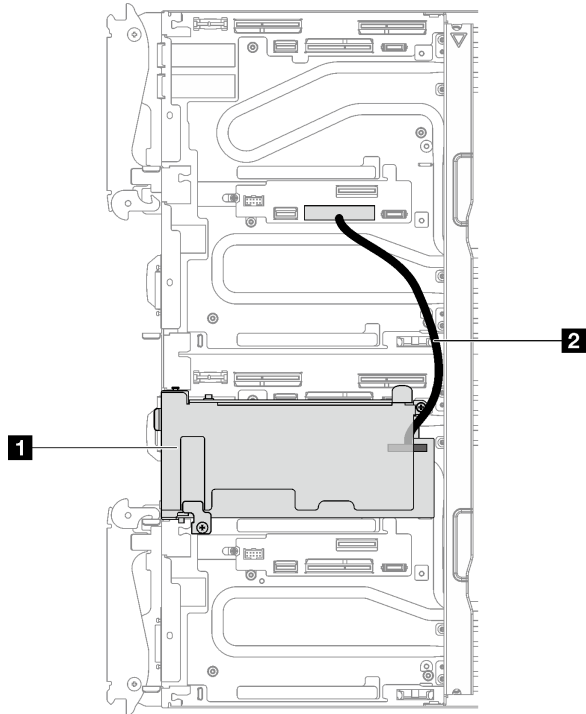
图 242. ConnectX-7 NDR 200/ConnectX-7 NDR 400 的共享 I/O 配置
