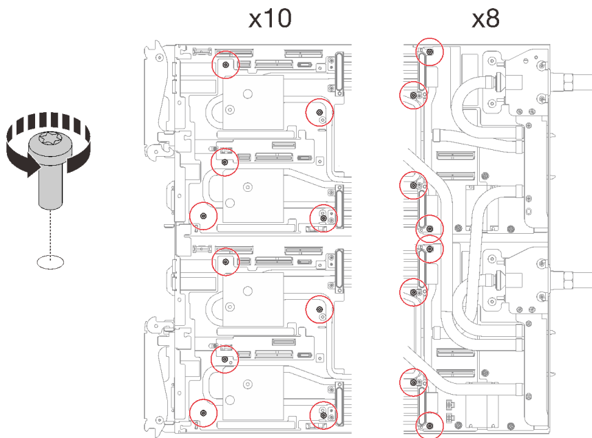
图 24. 卸下水循环模块螺钉
