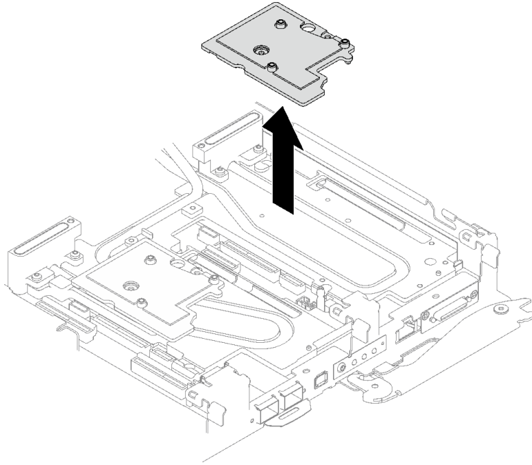
图 182. 卸下接口板
