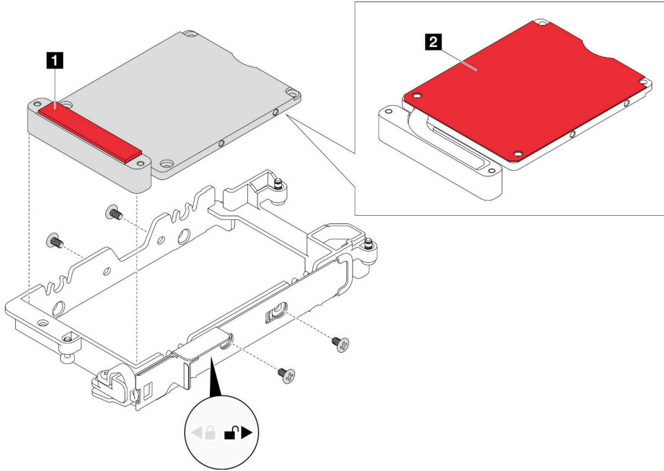
图 72. 安装导电板
