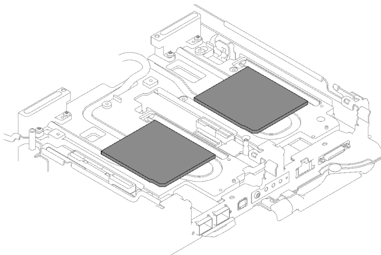
图 96. 间隙垫位置
