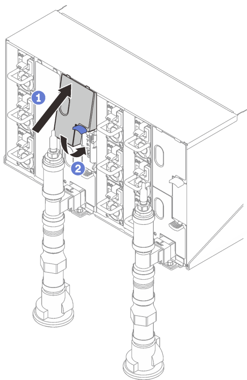
图 261. 安装上方 EMC 保护罩
