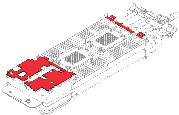
图 42. 水循环模块间隙垫
