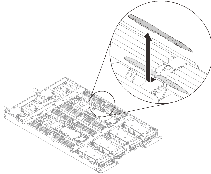
图 140. 卸下内存条工具
