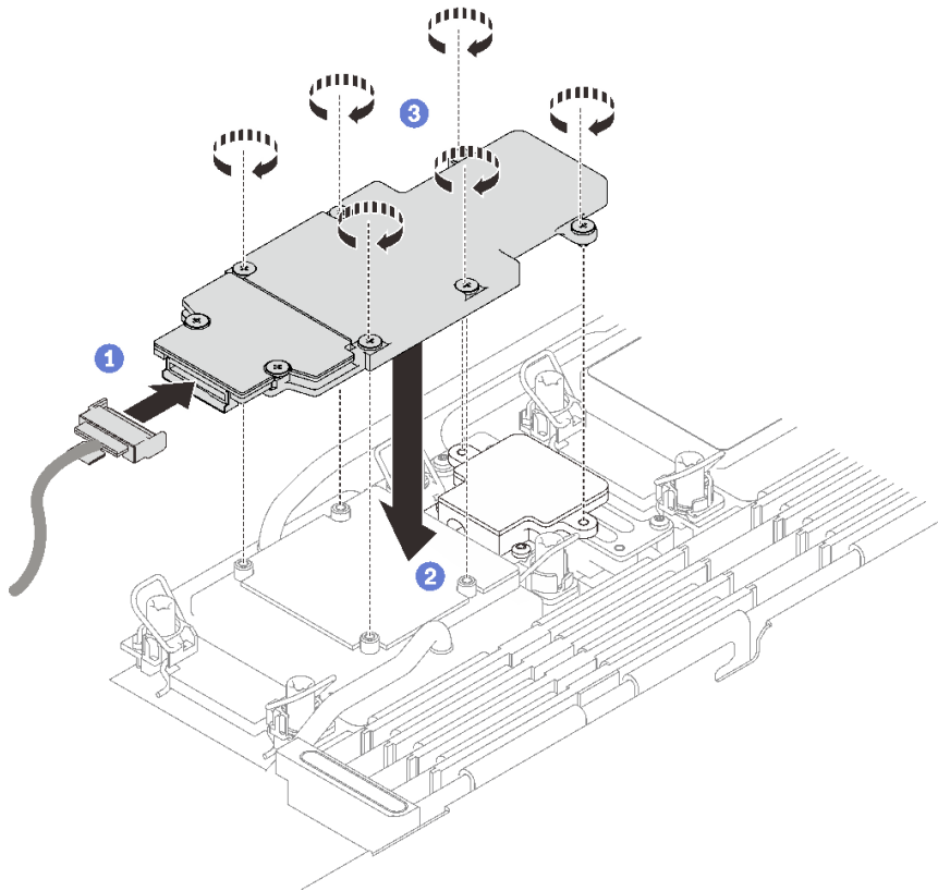
图 129. 安装 M.2 背板组合件
