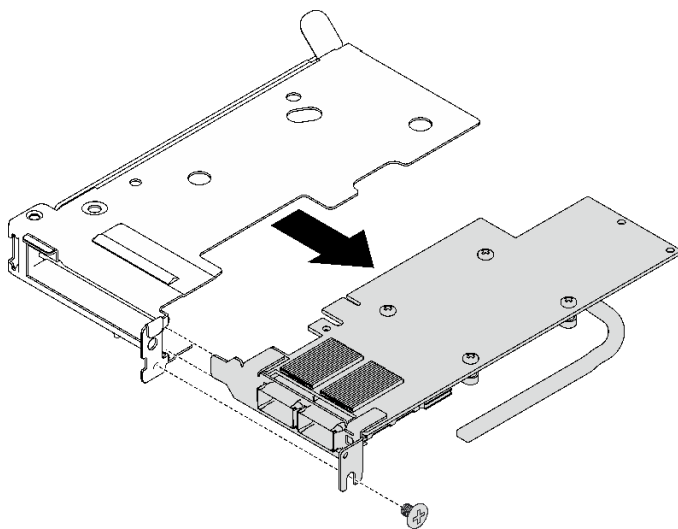
图 145. 卸下 PCIe 适配器
