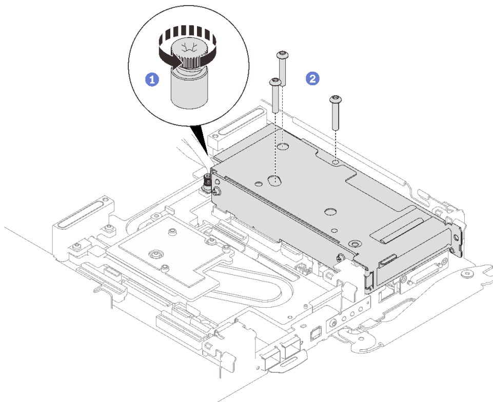
图 176. 卸下 PCIe 转接卡组合件
