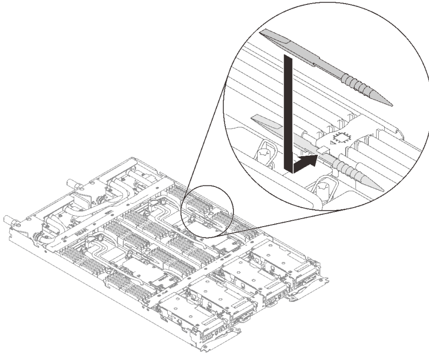
图 138. 安装内存条工具
