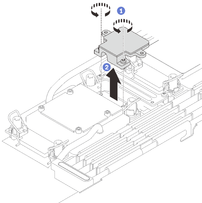
图 125. 卸下 M.2 背板冷却板
