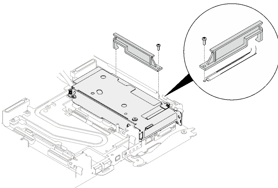
图 162. 安装导热管架
