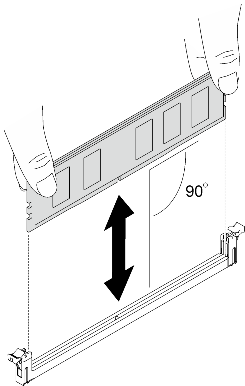
图 137. 卸下内存条
