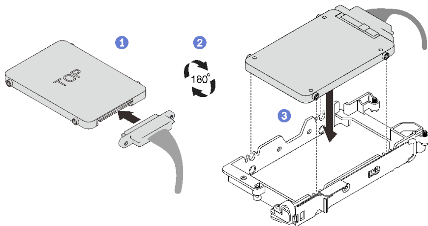
图 73. 安装下方硬盘
