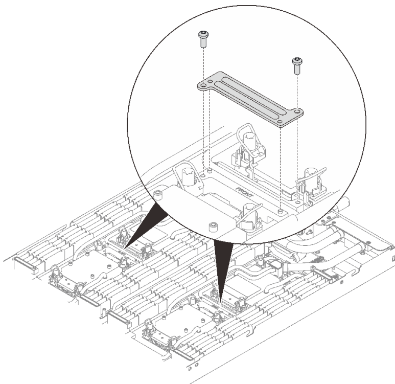
图 51. 安装 VR 夹板
