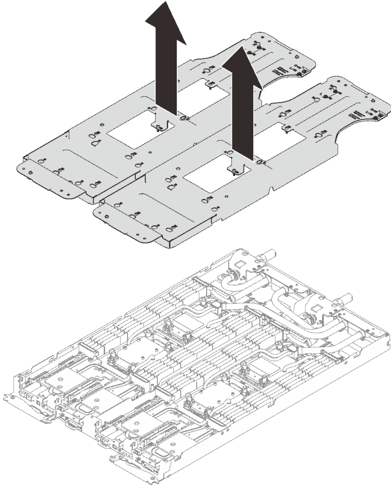
图 48. 卸下水循环模块载板
