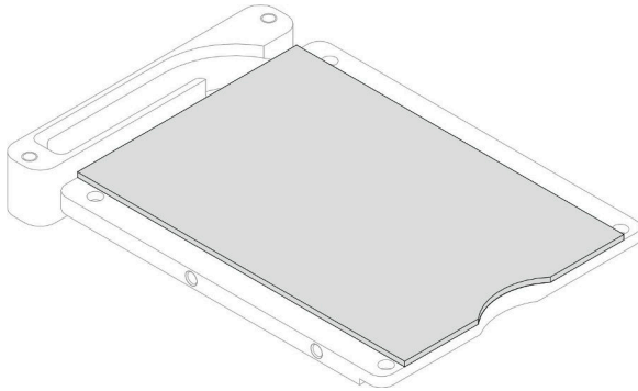
图 89. 安装导电板间隙垫
