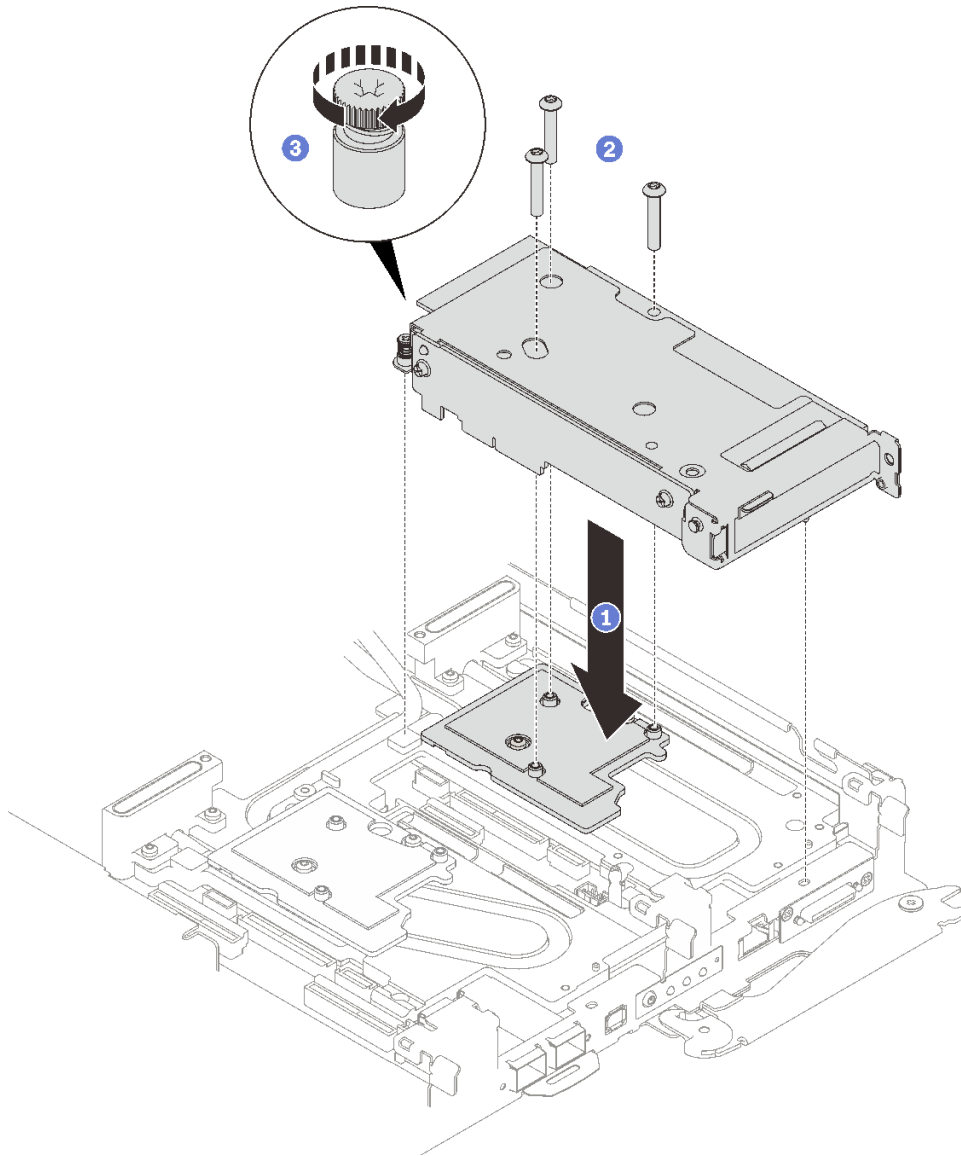
图 188. 安装 PCIe 转接卡组合件
