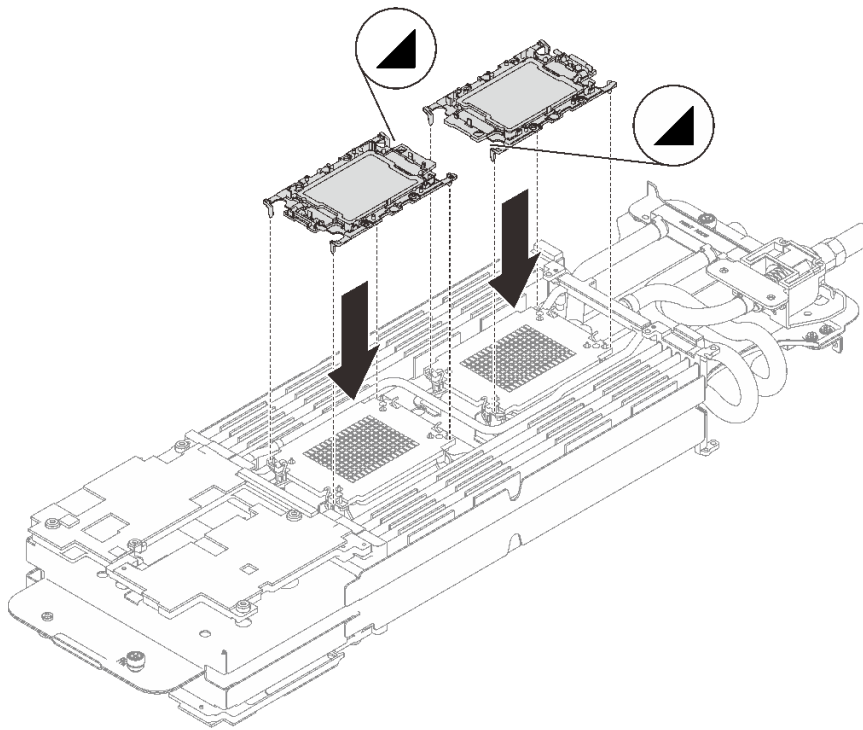
图 40. 安装处理器
