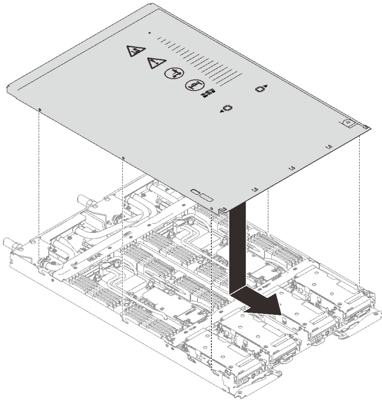
图 19. 安装托盘外盖
