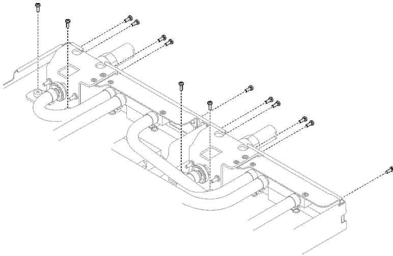
图 23. 卸下快接件螺钉
