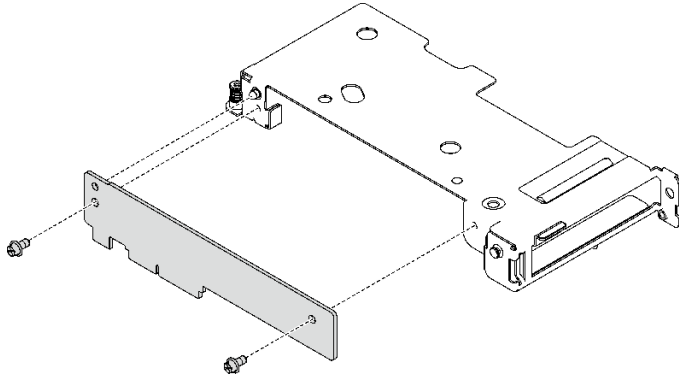
图 170. 卸下扩展板
