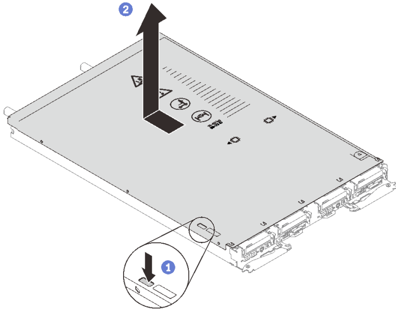
图 18. 卸下托盘外盖
