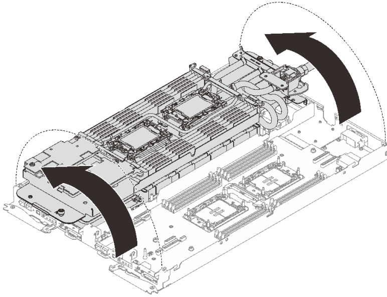
图 28. 折叠水循环模块
