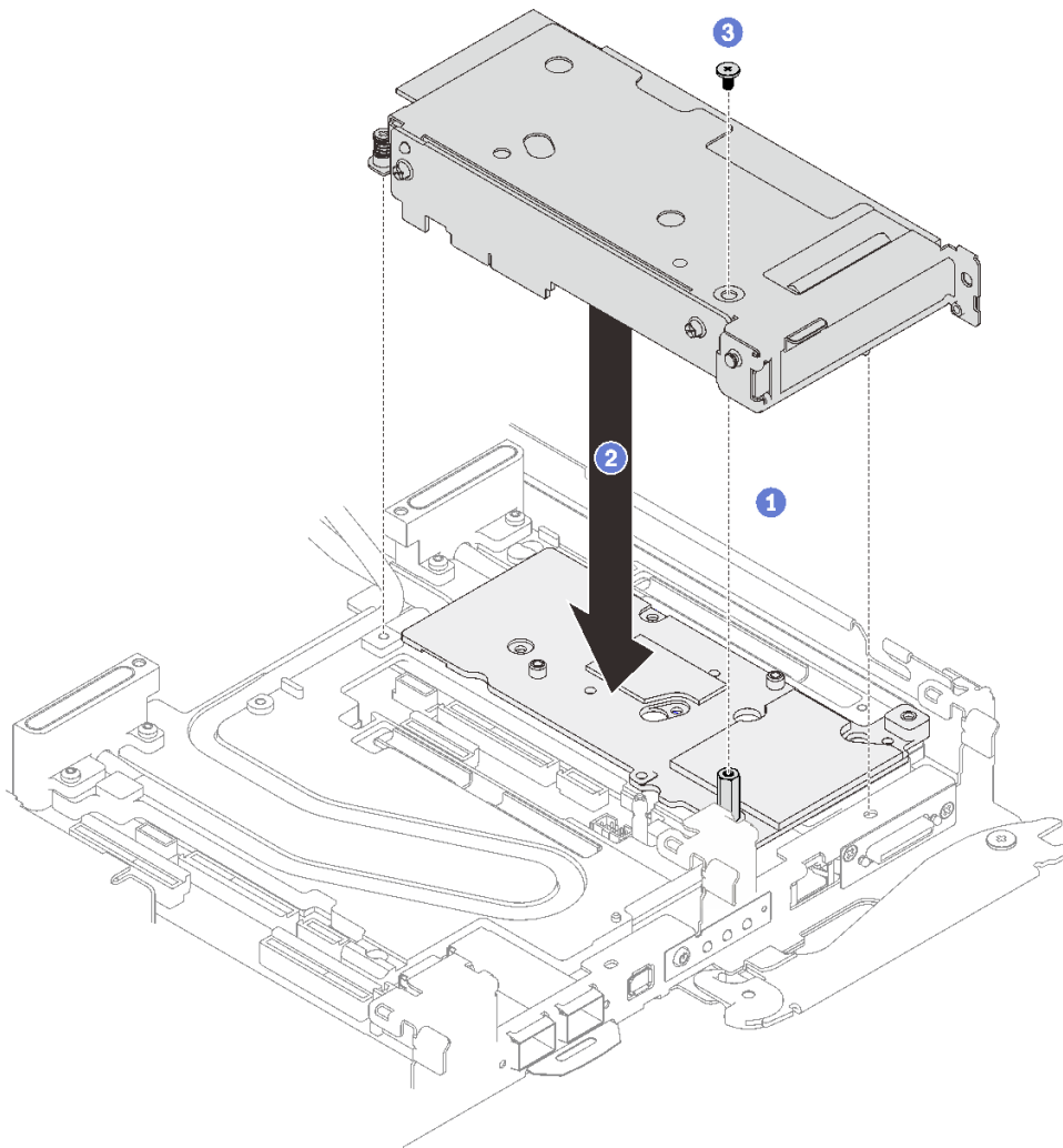
图 174. 安装 PCIe 转接卡组合件
