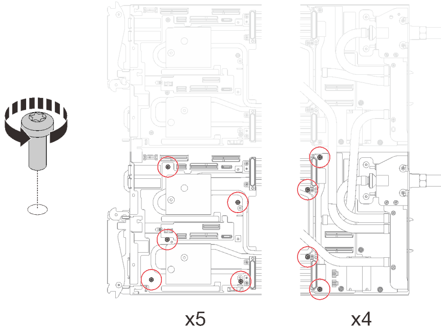
图 208. 卸下水循环模块螺钉
