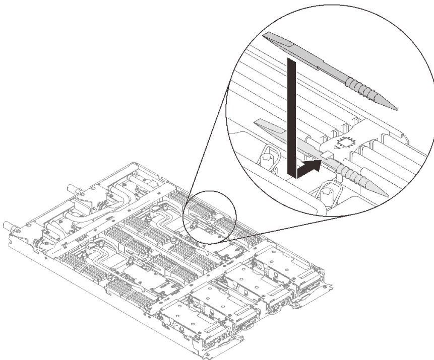
图 59. 安装内存条工具
