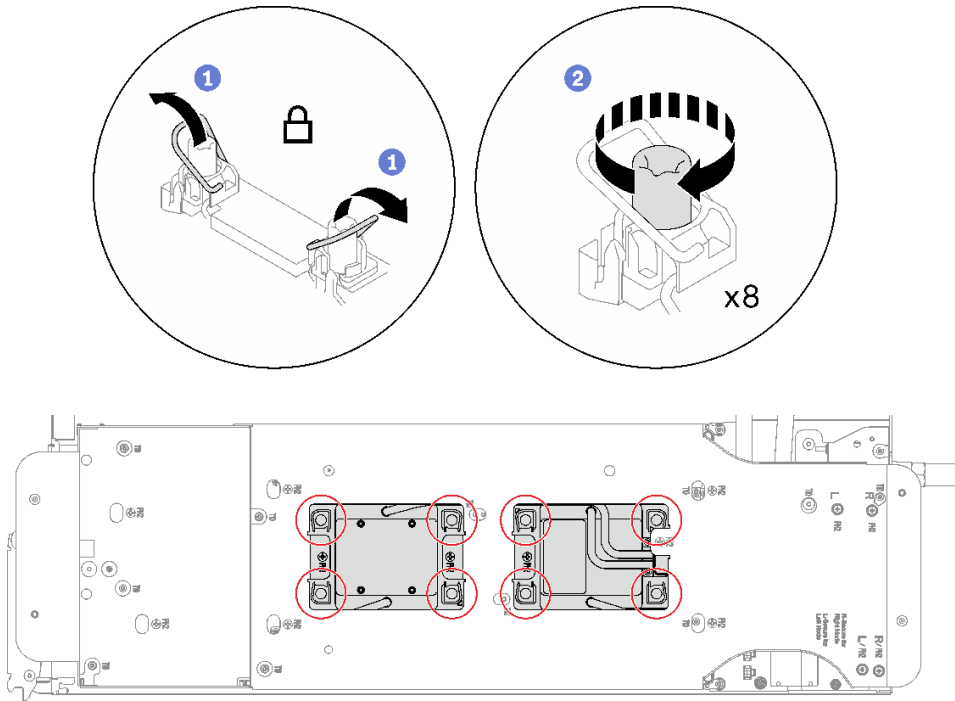
图 200. 安装处理器
