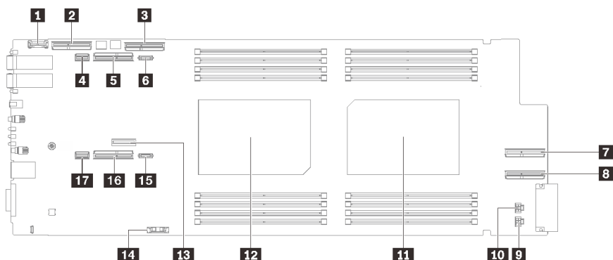
图 5. 计算节点主板上的内部接口
