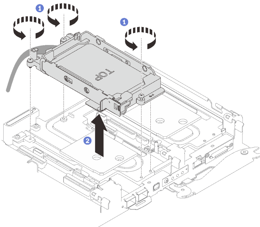
图 62. 卸下单 7 毫米硬盘仓组合件
