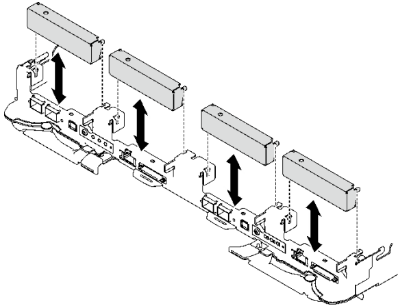
图 93. 安装空挡板填充件
