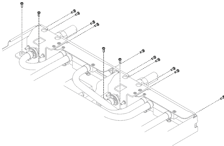
图 50. 安装快接件螺钉
