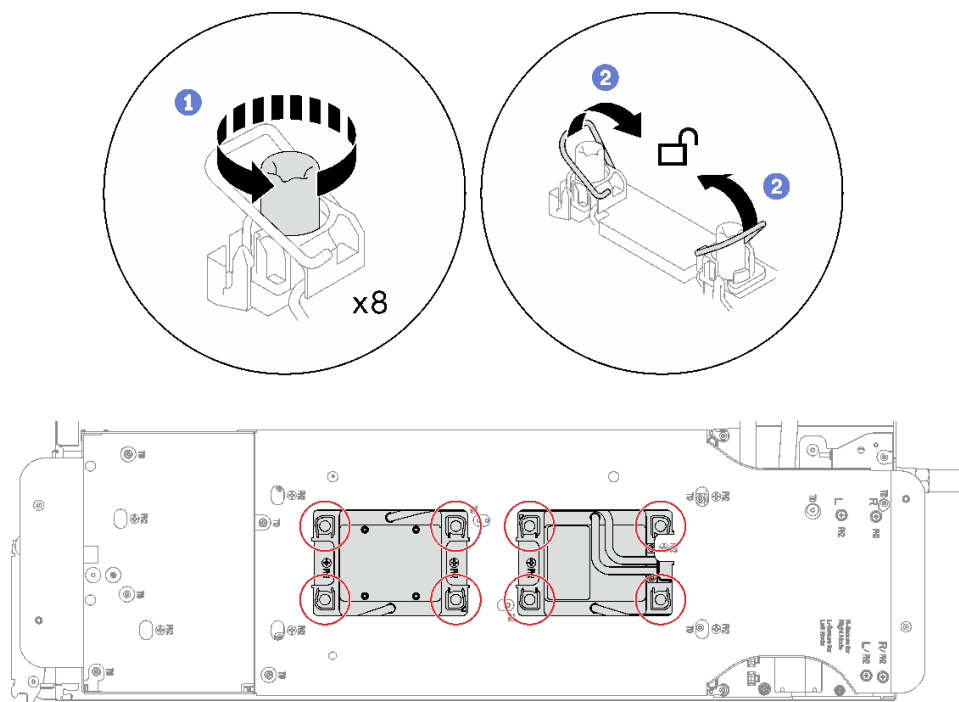
图 194. 松开处理器
