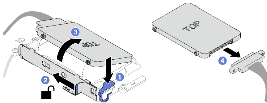
图 67. 卸下上方硬盘
