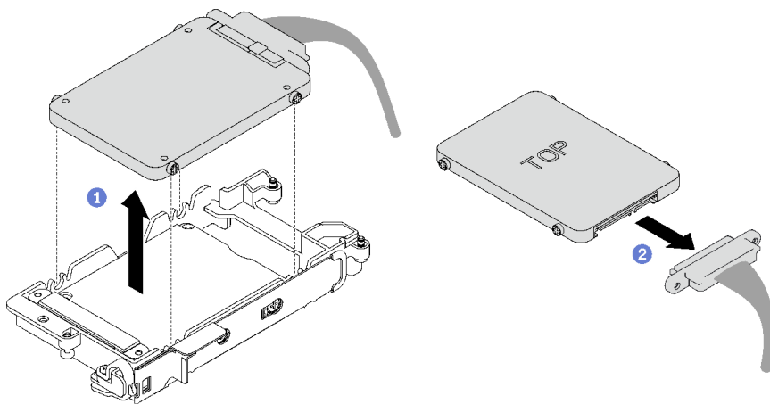
图 65. 卸下 7 毫米硬盘
