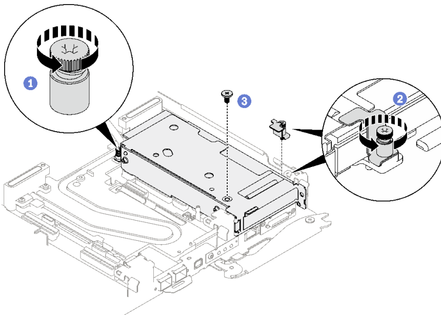
图 152. 卸下夹持支架的松不脱螺钉
