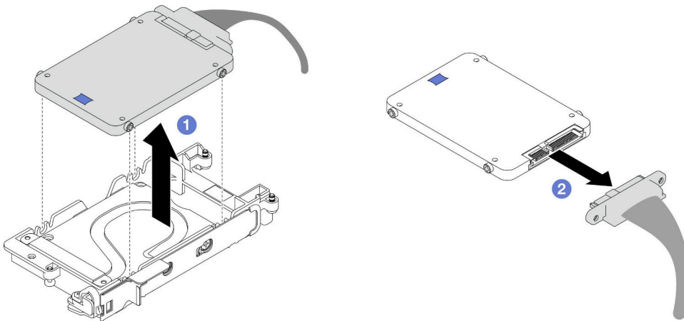
图 88. 卸下下方硬盘
