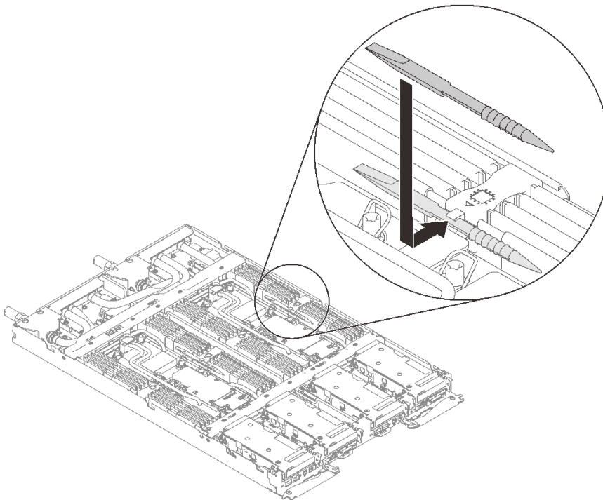
图 144. 安装内存条工具
