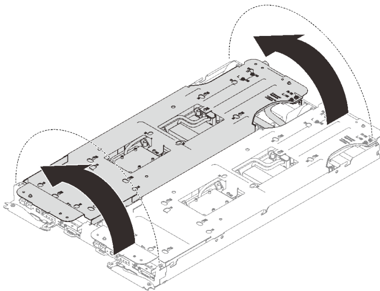
图 45. 展开水循环模块
