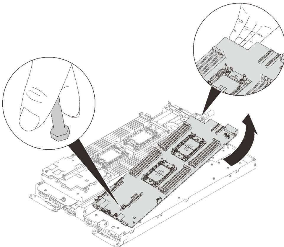
图 235. 卸下主板
