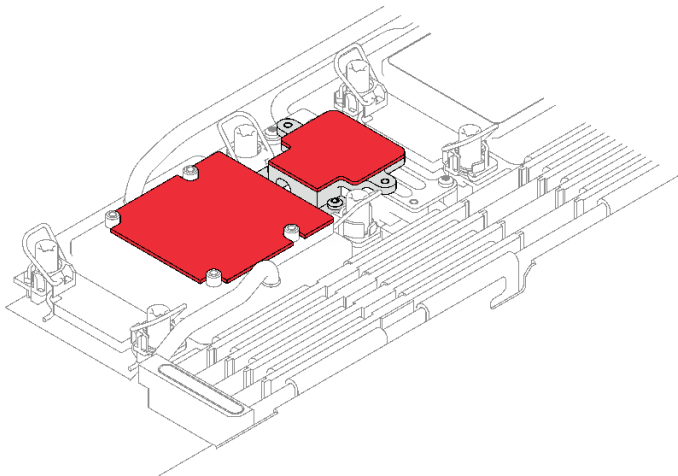
图 128. 处理器冷却板和 M.2 背板冷却板上的间隙垫
