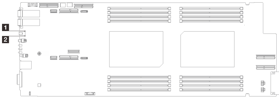
图 257. 主板 LED
