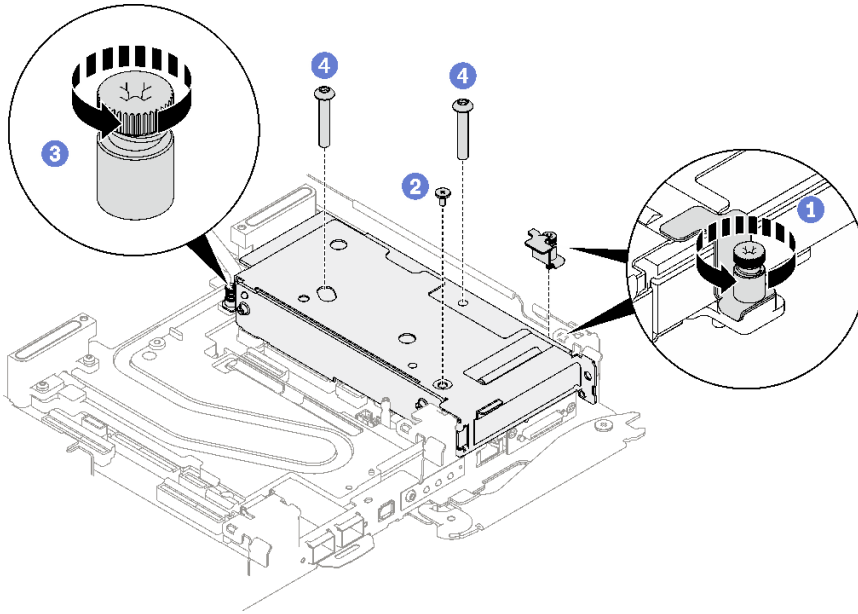
图 163. 卸下来持支架的松不脱螺钉
