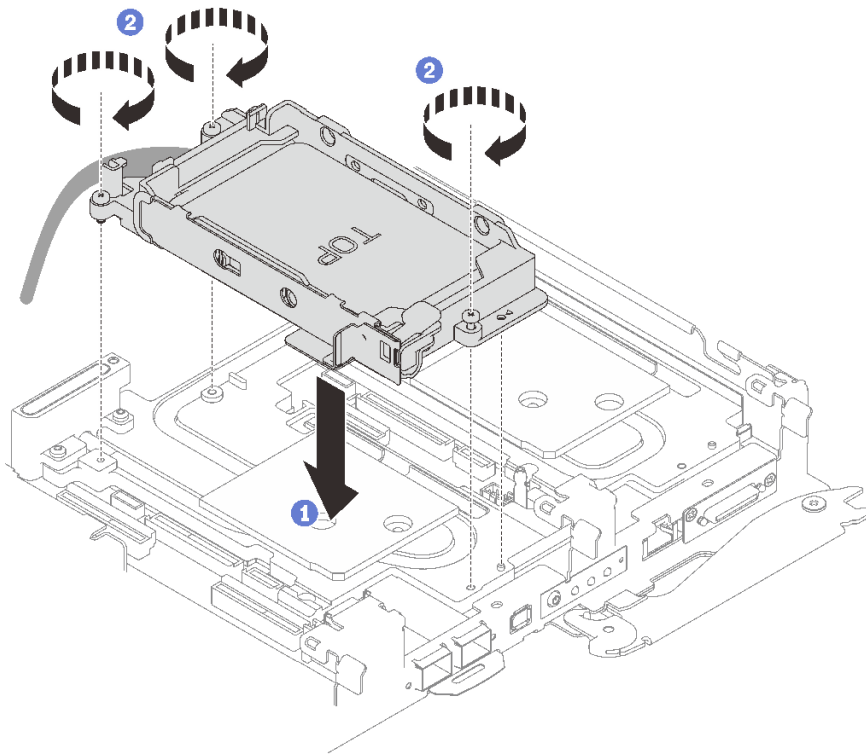
图 81. 安装单 7 毫米硬盘仓组合件
