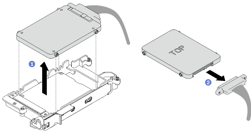
图 68. 卸下下方硬盘
