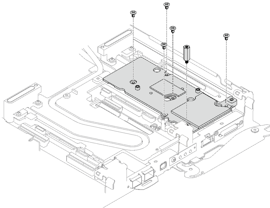
图 165. 卸下接口板
