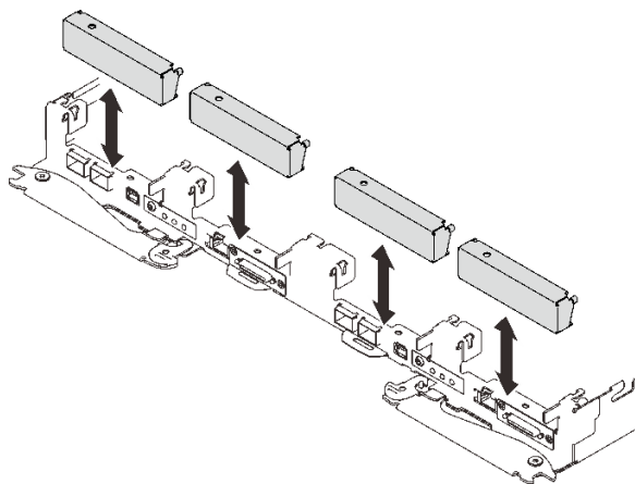
图 185. 卸下空挡板填充件
