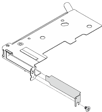
图 148. 卸下填充件
