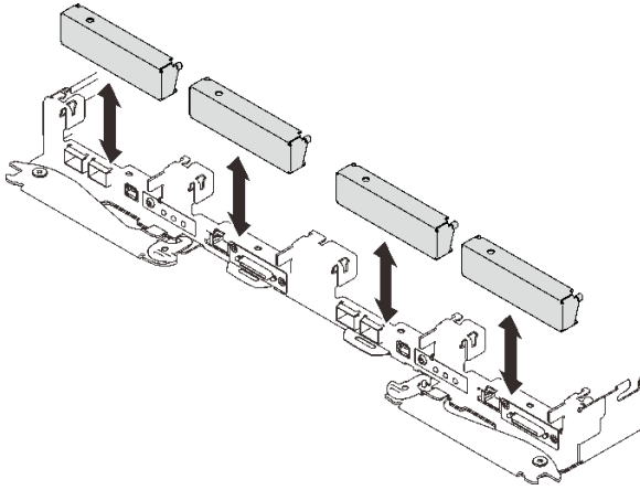
图 157. 卸下空挡板填充件
