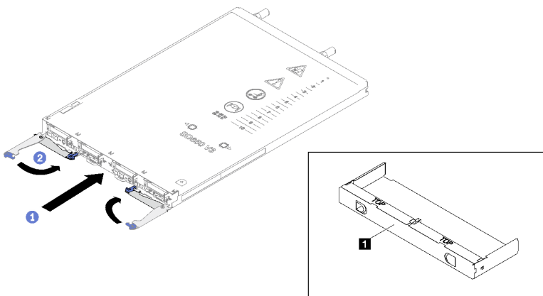
图 17. 安装托盘
