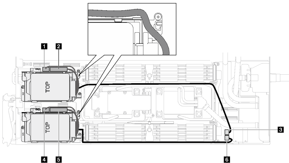
图 83. 硬盘组合件线缆布放
