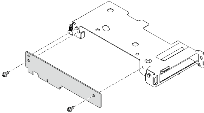
图 184. 卸下扩展板
