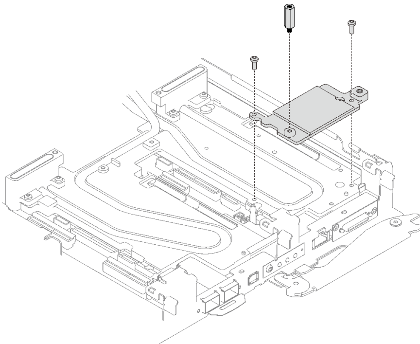
图 154. 卸下接口板
