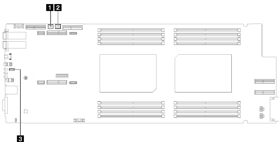
图 7. 计算节点主板上的开关
