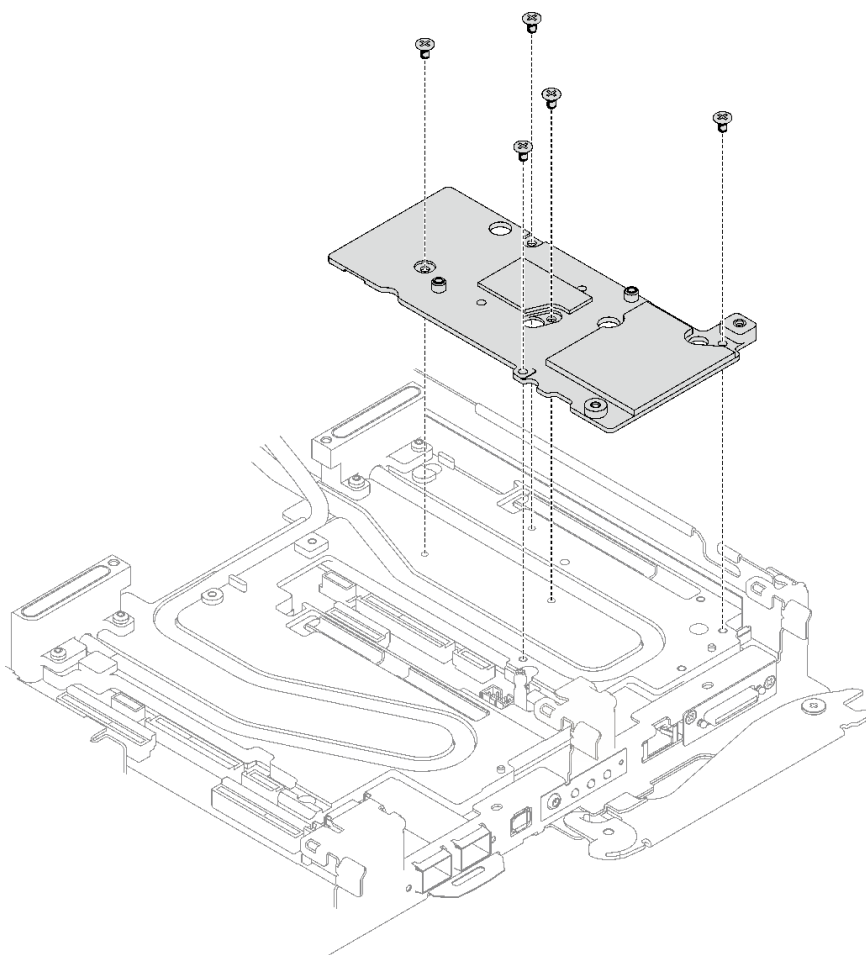
图 172. 安装接口板
