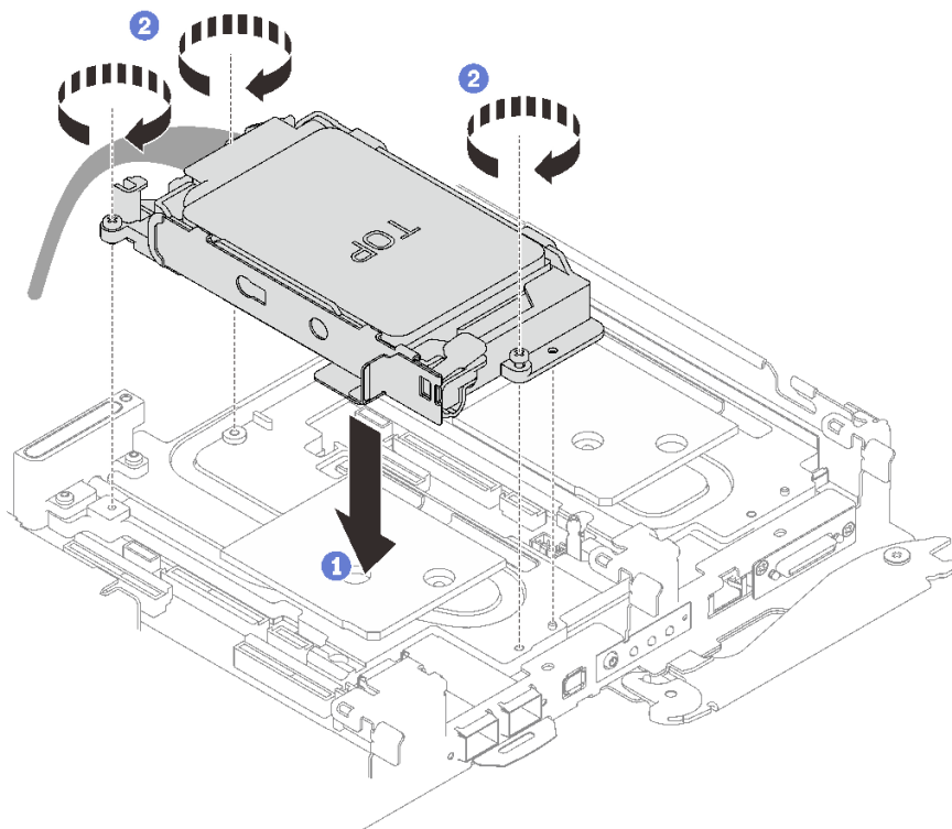
图 82. 安装双 7 毫米硬盘仓组合件
