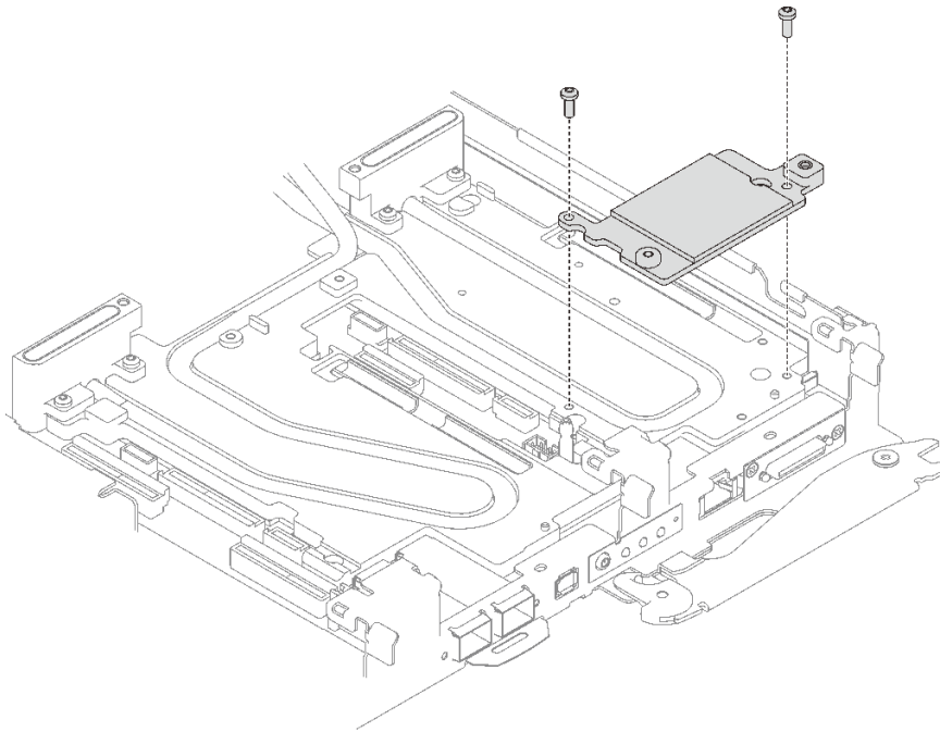
图 158. 安装接口板
