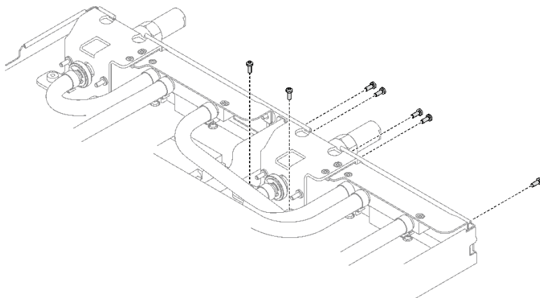
图 191. 卸下快接件螺钉
