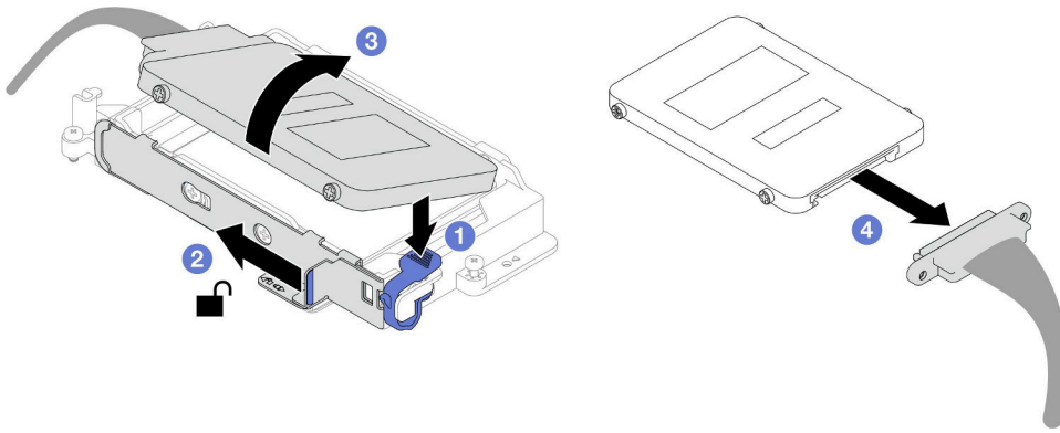
图 87. 卸下上方硬盘 (7 毫米 NVMe)
