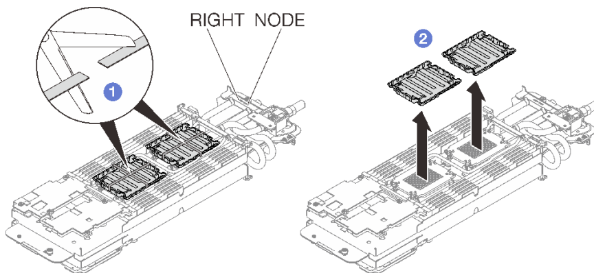
图 222. 卸下塑料油脂外盖
