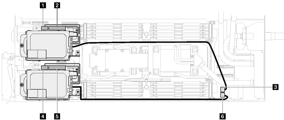
图 120. E3.S 硬盘线缆布放
