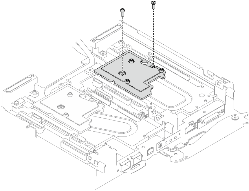
图 179. 卸下接口板
