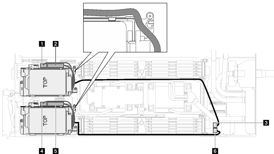
图 84. 硬盘组合件线缆布放
