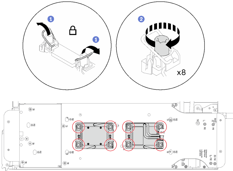
图 227. 安装处理器
