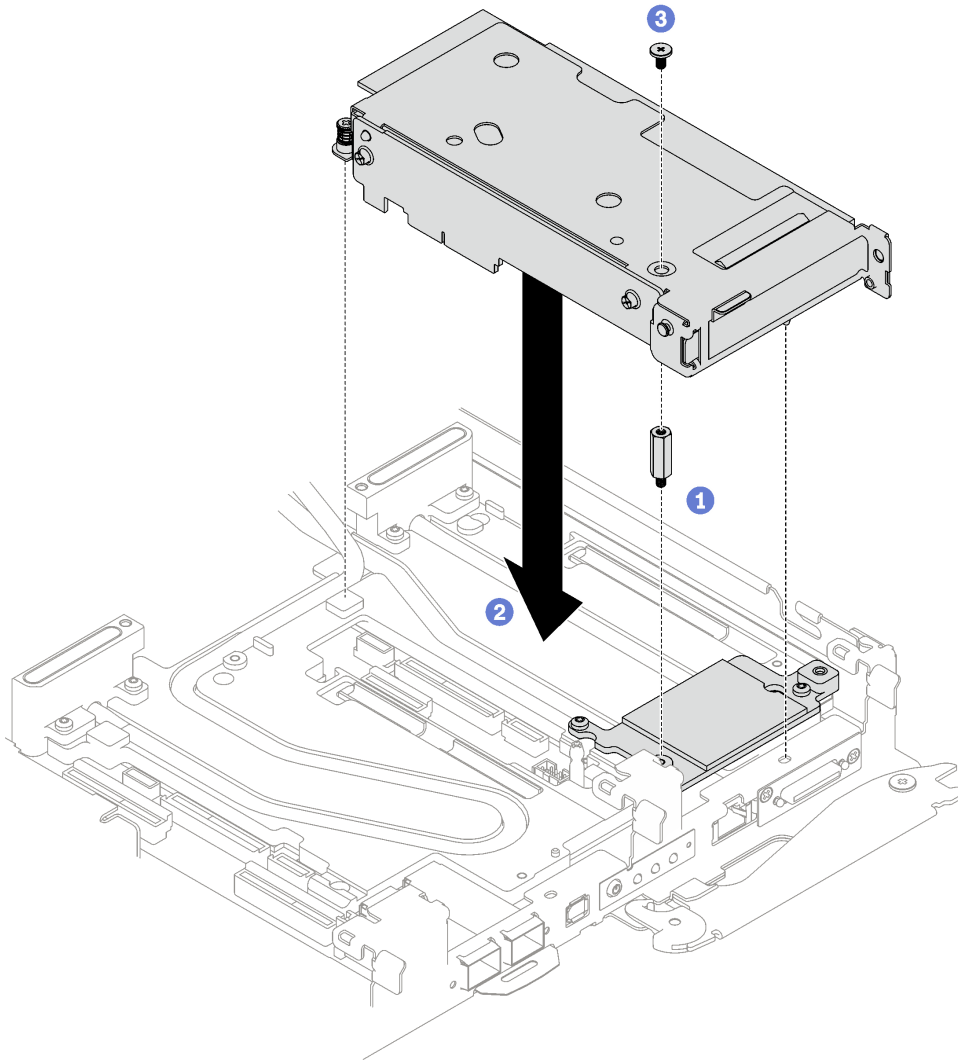
图 160. 安装 PCIe 转接卡组合件
