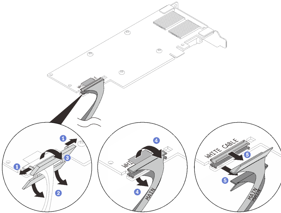
图 146. 拔下 PCIe 适配器线缆
