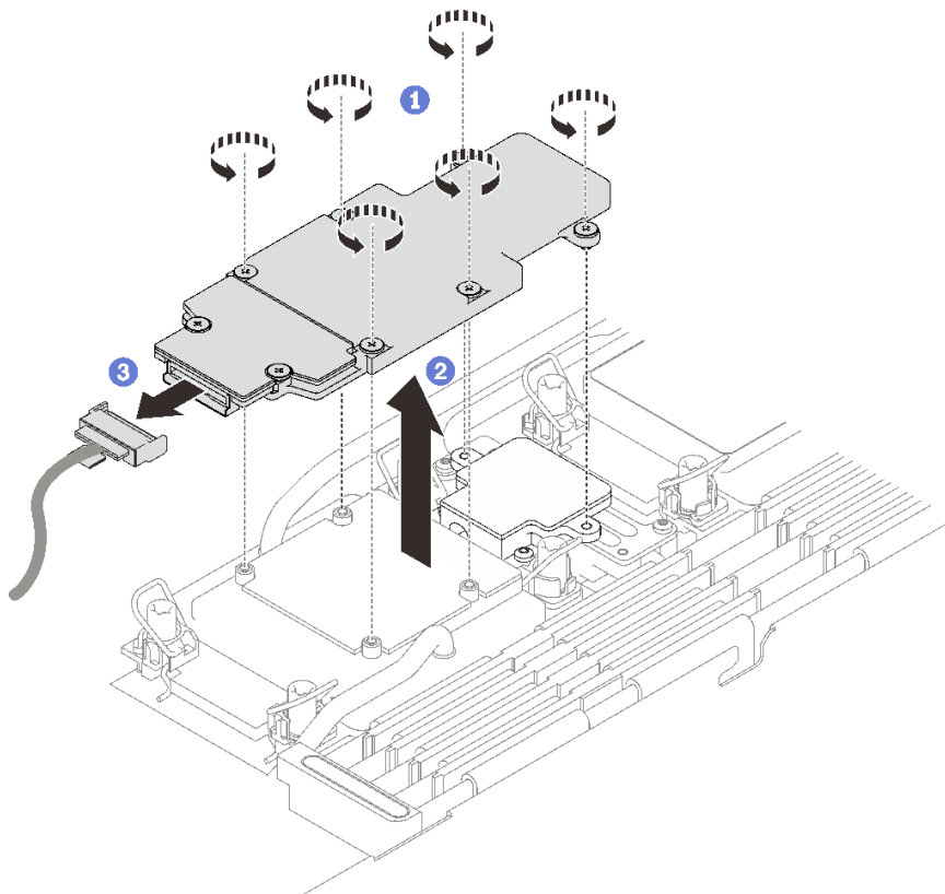
图 124. 卸下 M.2 背板组合件
