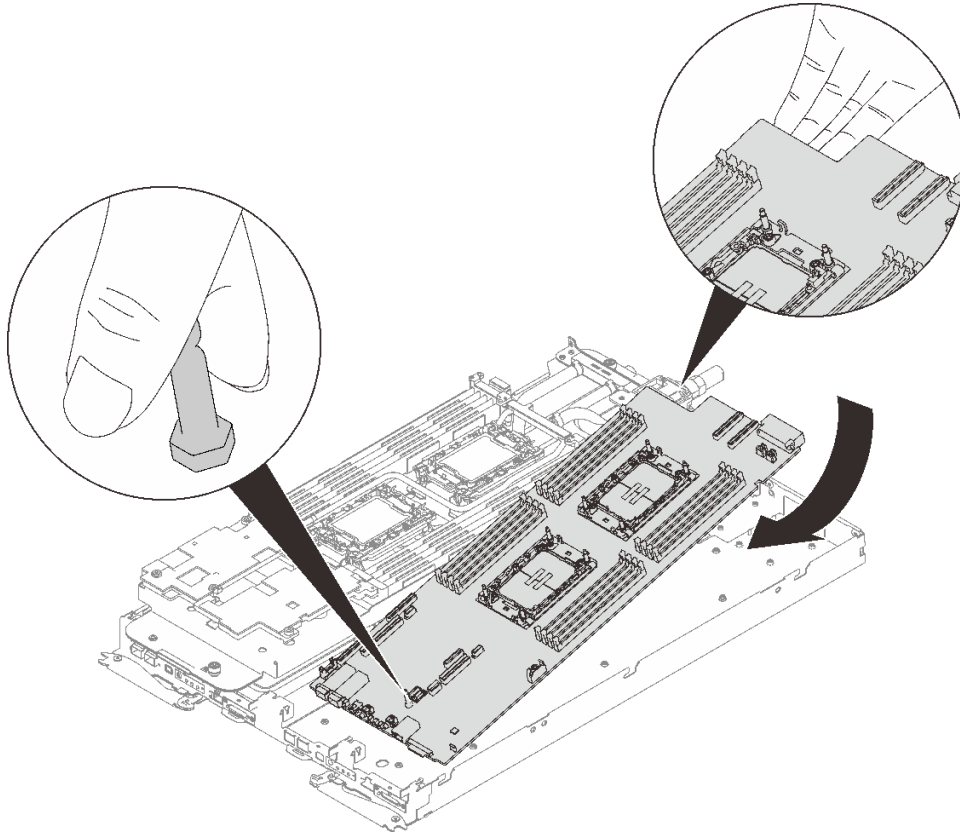
图 237. 安装主板
