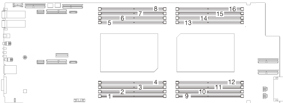
图 134. 内存条插槽位置
