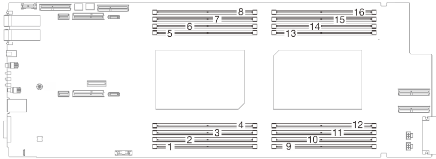
图 14. 内存条和处理器布局
