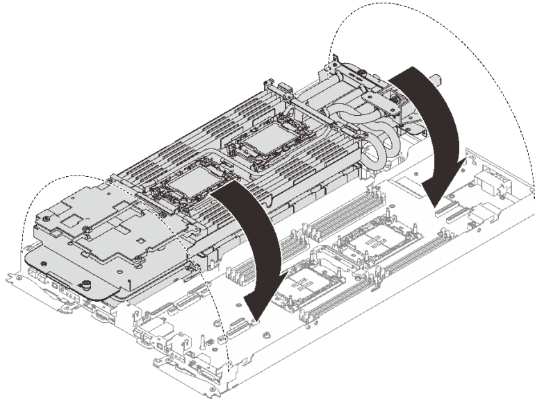
图 226. 安装水循环模块
