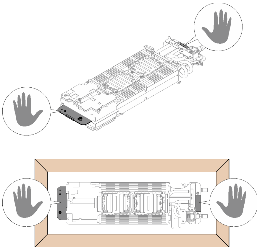
图 38. 从包装盒中取出水循环模块时的操作点
