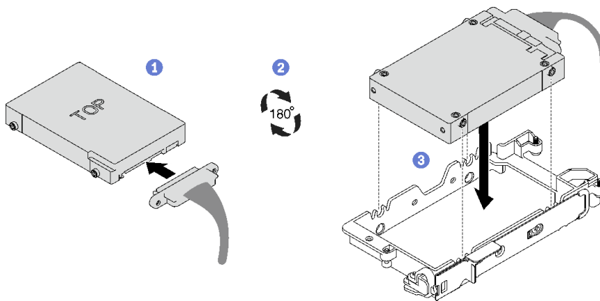
图 71. 安装 15 毫米硬盘
