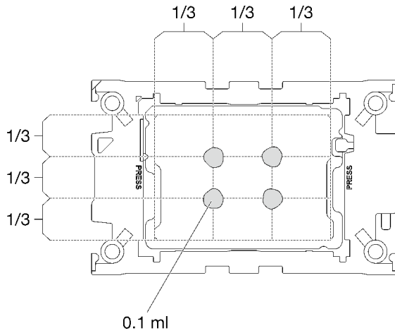
图 218. 涂抹导热油脂
