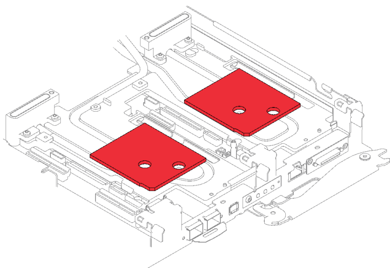
图 79. 间隙垫位置
