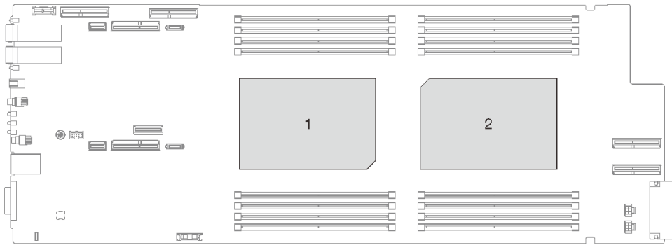
图 217. 处理器位置
