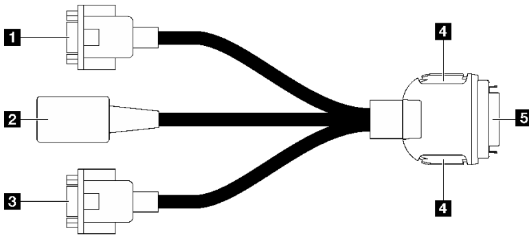
图 4. KVM 分支线缆上的接口和组件
