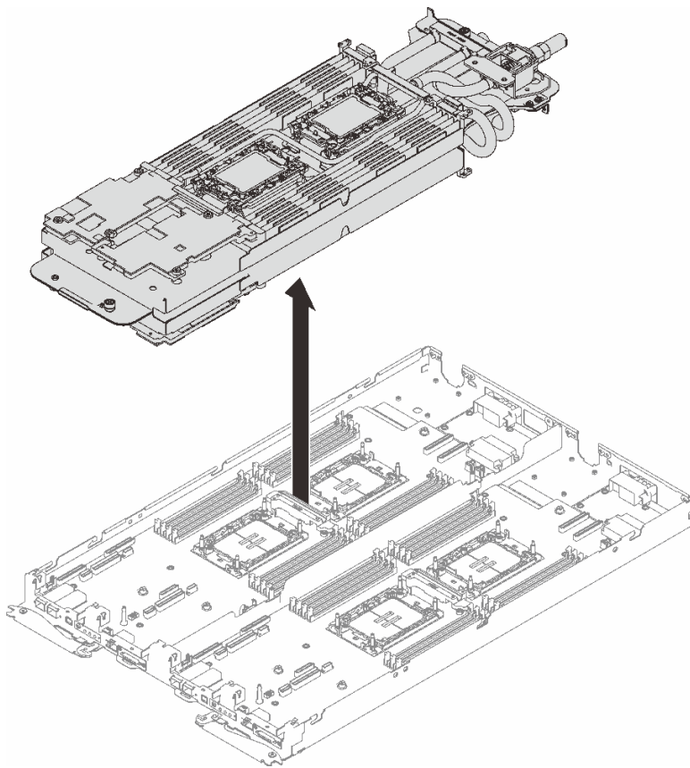
图 33. 卸下水循环模块
