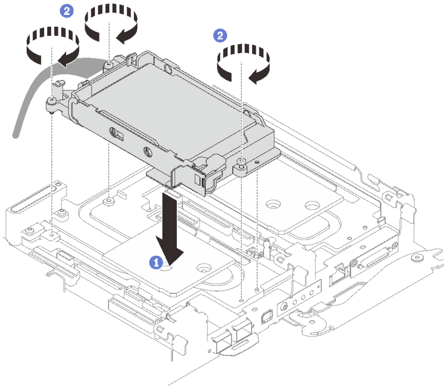
图 80. 安装单 15 毫米硬盘仓组合件
