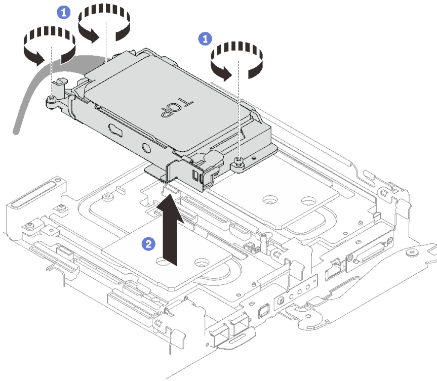
图 63. 卸下双 7 毫米硬盘仓组合件
