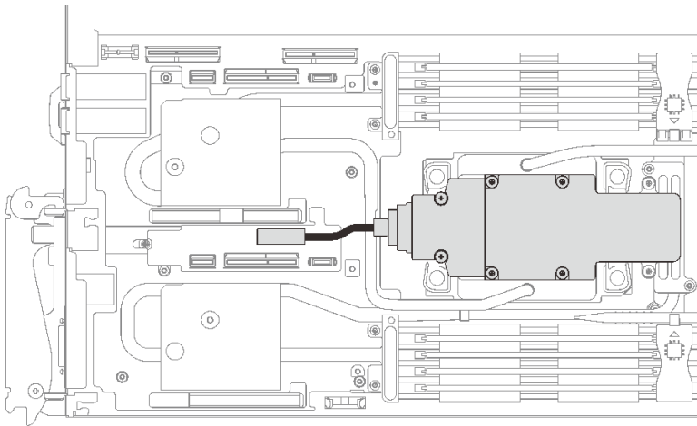
图 123. 拔下 M.2 背板组合件线缆
