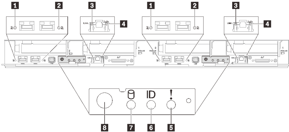
图 252. SD650 V3 托盘正面 LED
