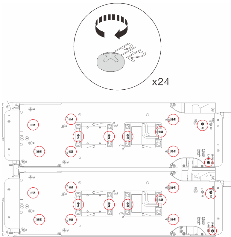
图 26. 安装水循环模块载板的螺钉
