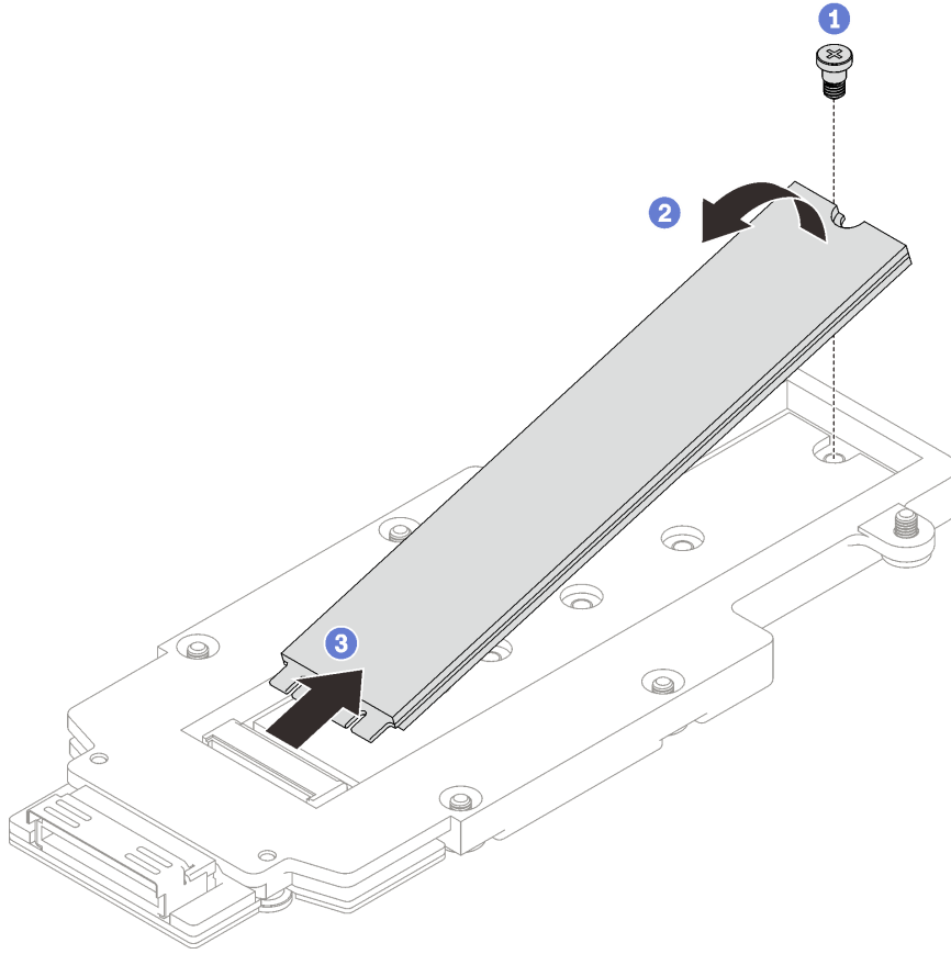
图 131. 卸下 M.2 硬盘
