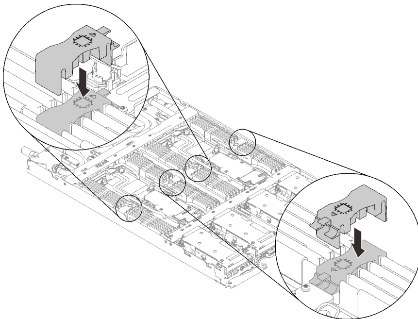
图 58. 安装 DIMM 梳
