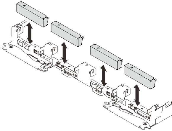
图 183. 安装空挡板填充件
