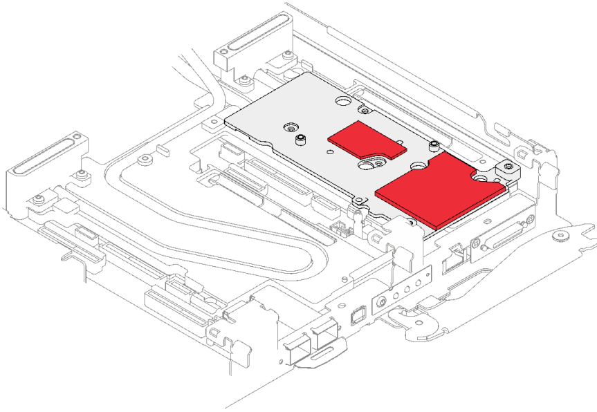
图 173. 适用于 CX-7 NDR 200 的接口板油灰垫
