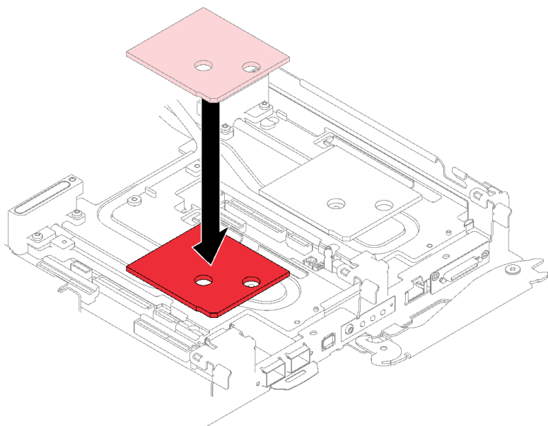
图 78. 更换间隙垫
