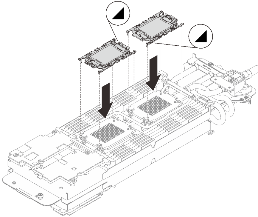
图 223. 安装处理器
