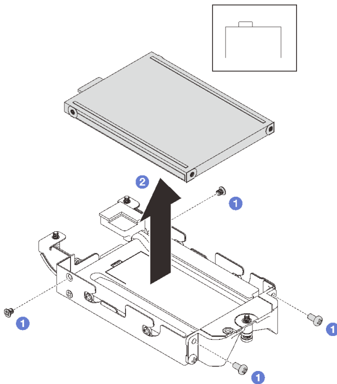
图 105. 卸下底部 E3.S 硬盘
