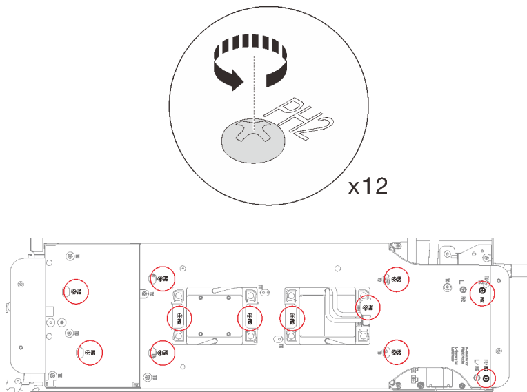
图 228. 拧松水循环模块载板的螺钉
