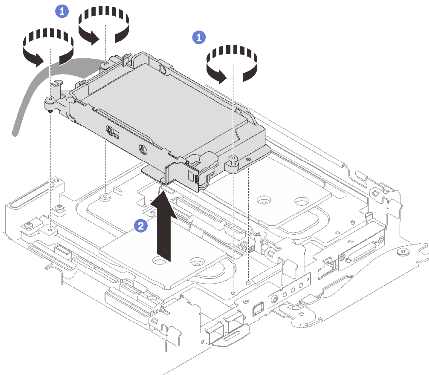
图 61. 卸下单 15 毫米硬盘仓组合件
