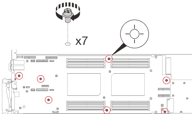
图 234. 卸下主板螺钉
