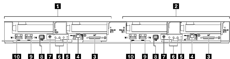
图 2. SD650 V3 托盘
