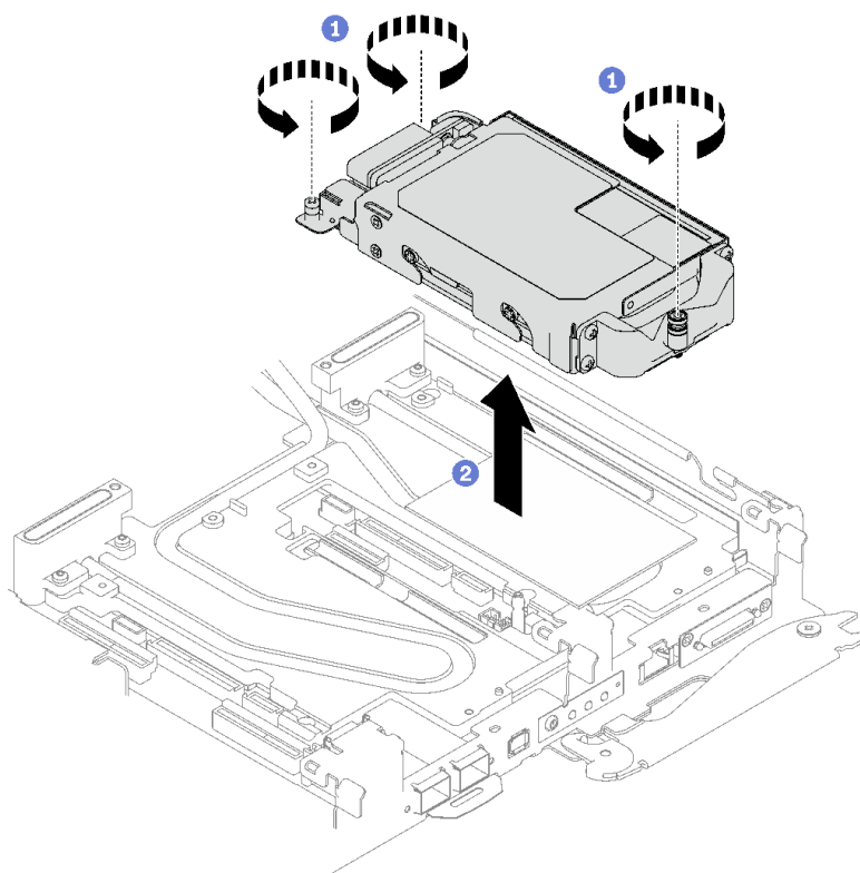
图 100. 卸下 E3.S 硬盘仓组合件
