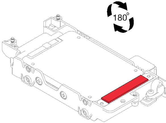
图 76. 间隙垫位置
