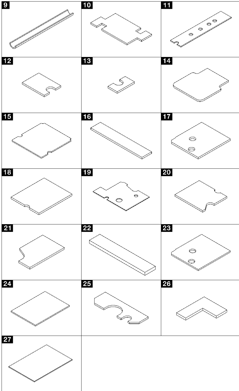
图 15. SD650 V3 中使用的间隙垫和油灰垫
