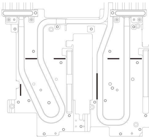
图 77. 水循环模块上的间隙垫对齐标记
