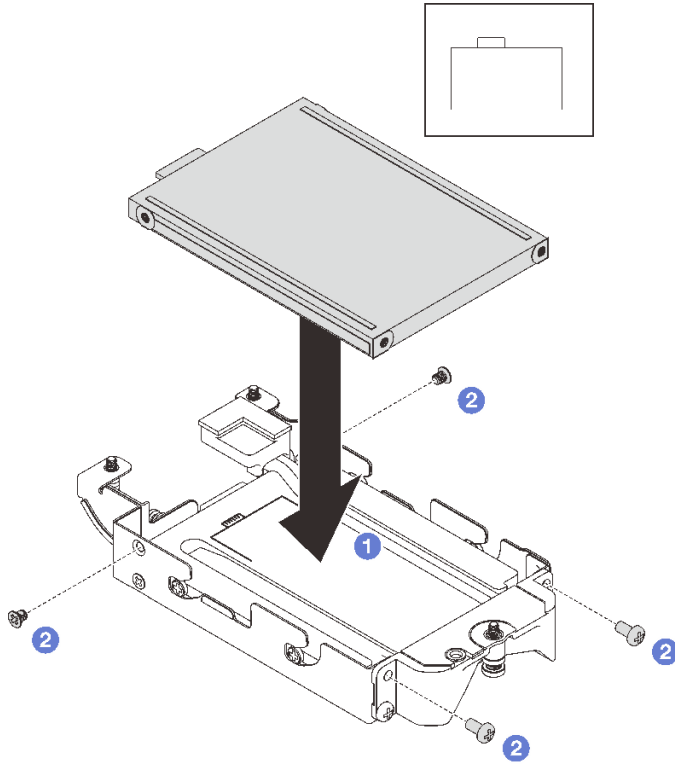
图 112. 安装底部 E3.S 硬盘
