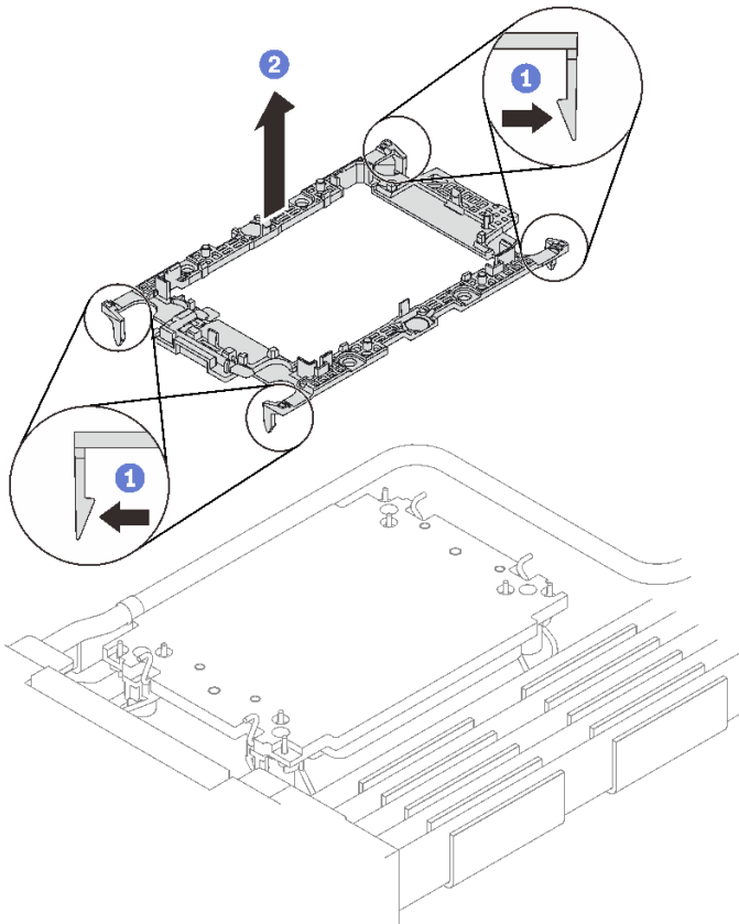
图 32. 卸下处理器固定器
