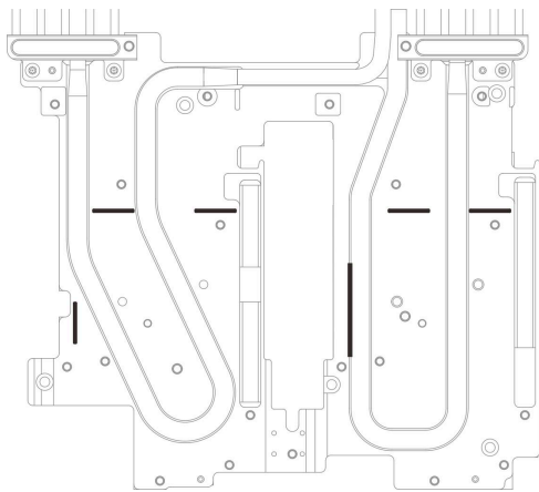
图 94. 水循环模块上的间隙垫对齐标记
