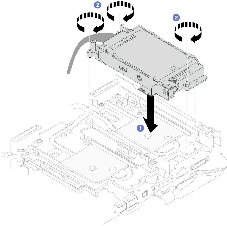
图 97. 安装 7 毫米 NVMe 硬盘仓组合件
