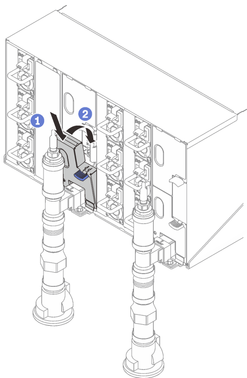
图 262. 安装下方 EMC 保护罩
