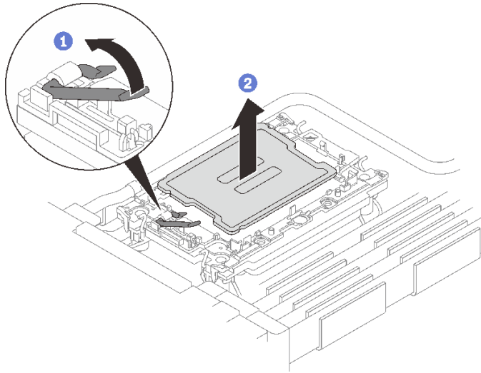
图 214. 卸下处理器
