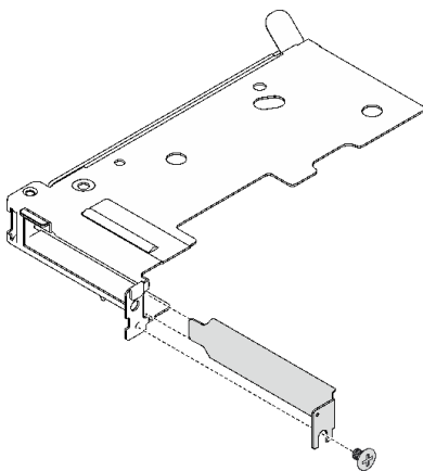
图 147. 安装填充件
