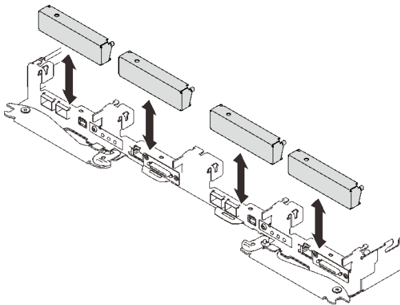
图 116. 安装空挡板填充件
