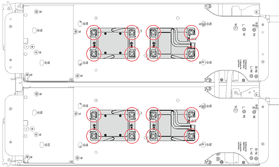
图 46. 拧紧内六角 T30 松不脱螺钉
