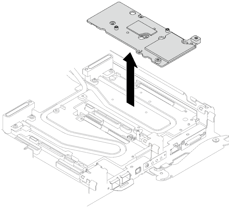
图 168. 卸下接口板
