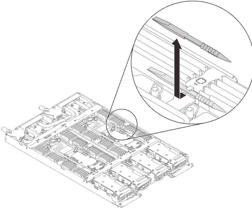
图 56. 卸下内存条工具
