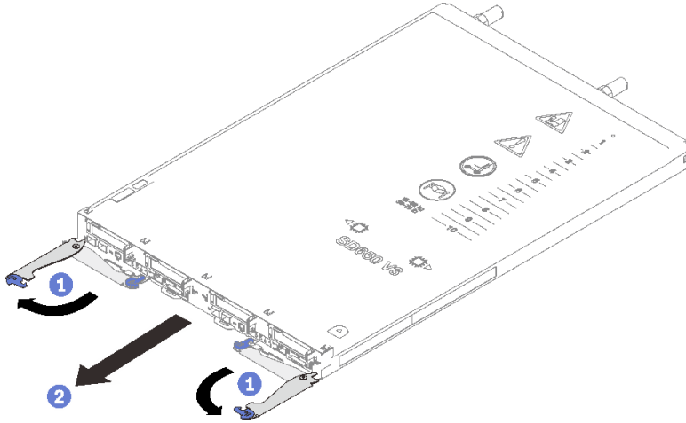
图 16. 卸下托盘
