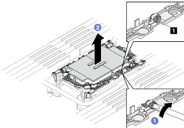
图 215. 卸下处理器 (Intel® Xeon® CPU Max 处理器)
