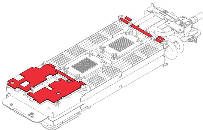
图 198. 水循环模块间隙垫
