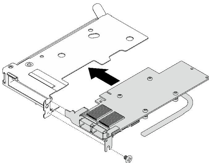
图 150. 安装 PCIe 适配器
