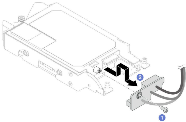
图 104. 卸下 E3.S 硬盘线缆端背板
