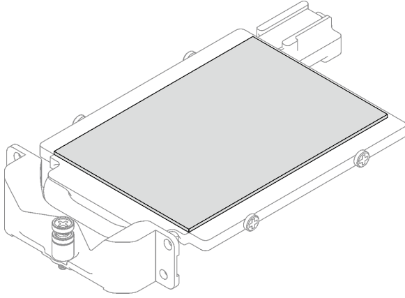
图 109. 更换导电板间隙垫
