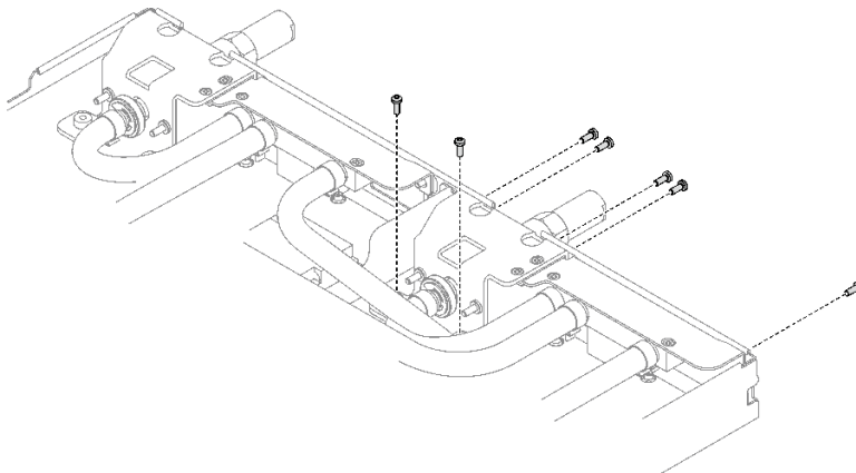
图 209. 卸下快接件螺钉
