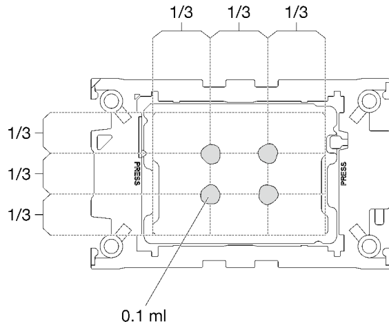
图 34. 涂抹导热油脂
