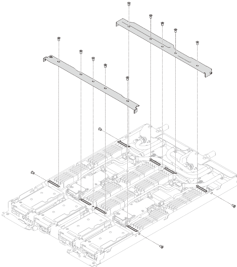
图 20. 卸下横梁 (SD650 V3)
