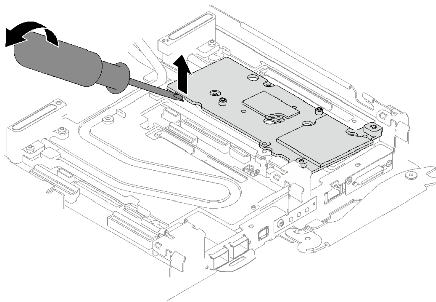
图 167. 将接口板从水循环模块冷却板上松开
