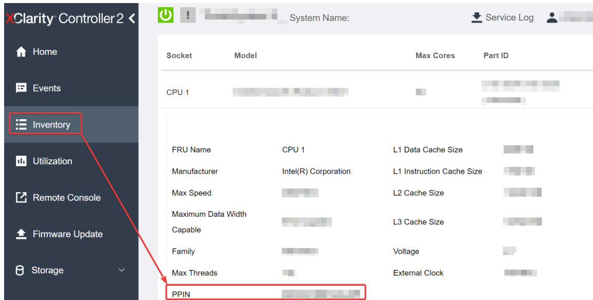
图 245. 通过 XCC Web GUI 读取 PPIN
