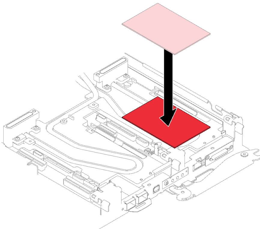
图 118. 更换间隙垫
