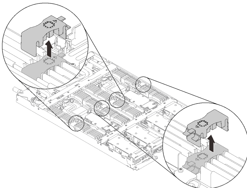
图 57. 卸下 DIMM 梳
