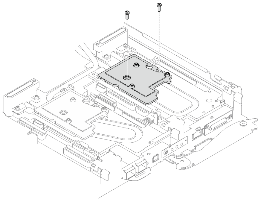
图 186. 安装接口板
