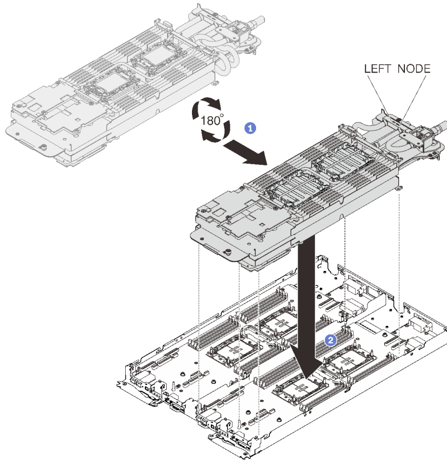
图 43. 安装水循环模块载板
