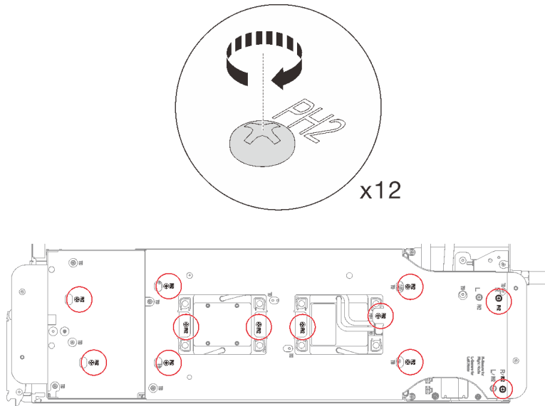
图 211. 安装水循环模块载板的螺钉
