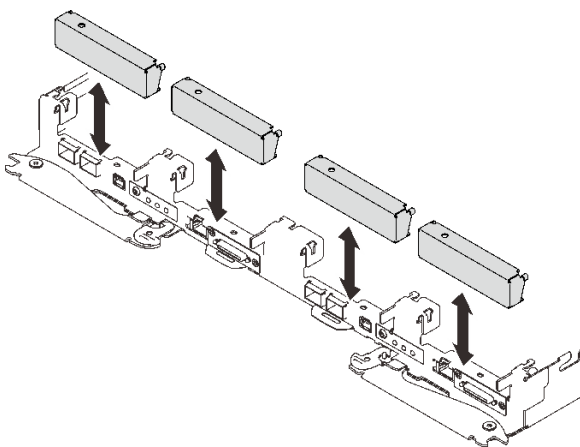
图 155. 安装空挡板填充件
