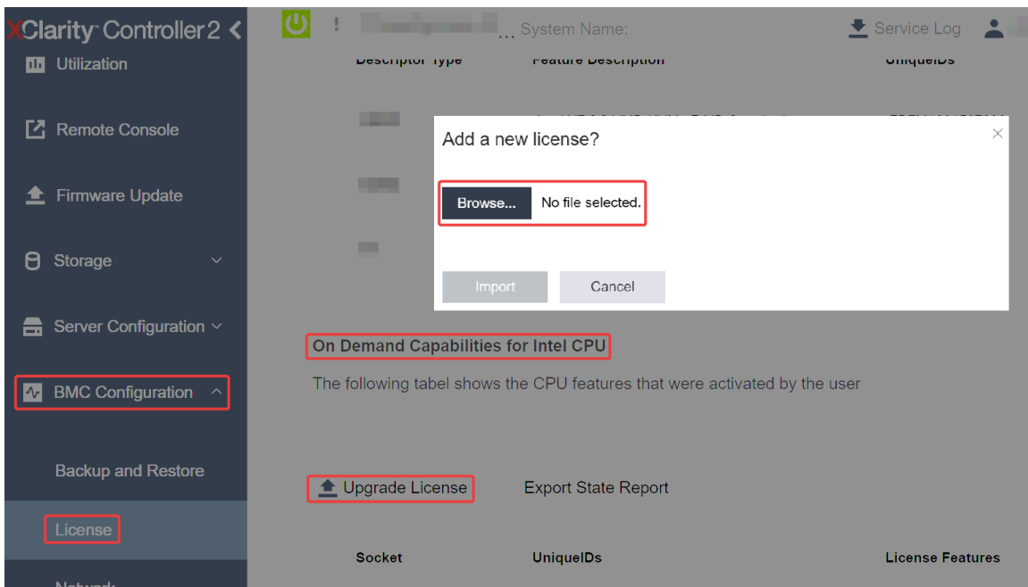
图 246. 通过 XCC Web GUI 上传激活密钥
