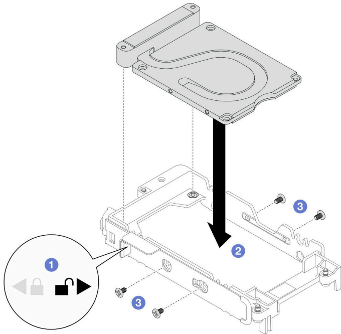
图 90. 安装导电板
