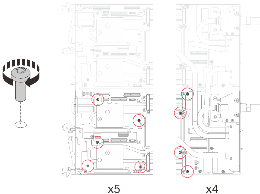
图 230. 安装水循环模块螺钉
