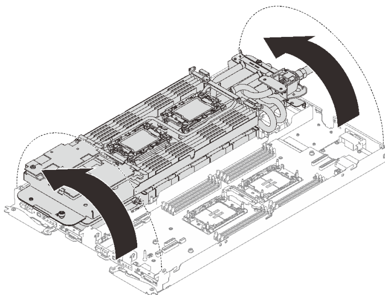
图 195. 折叠水循环模块
