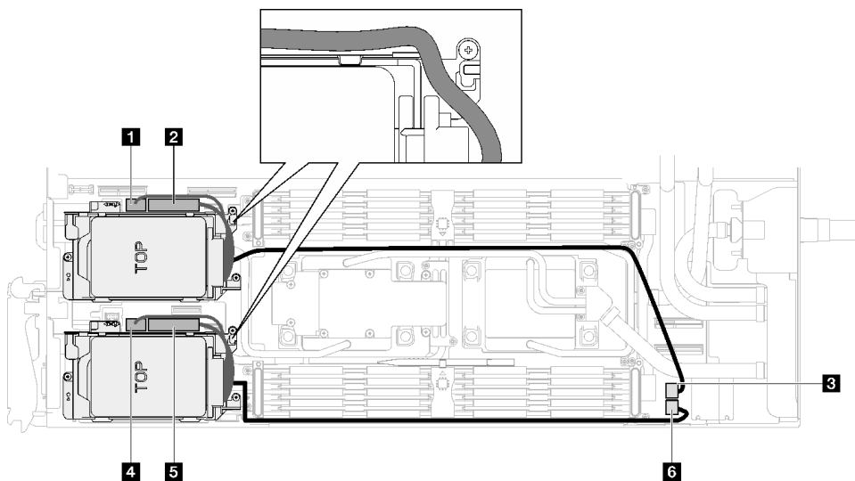
图 98. 硬盘组合件线缆布放
