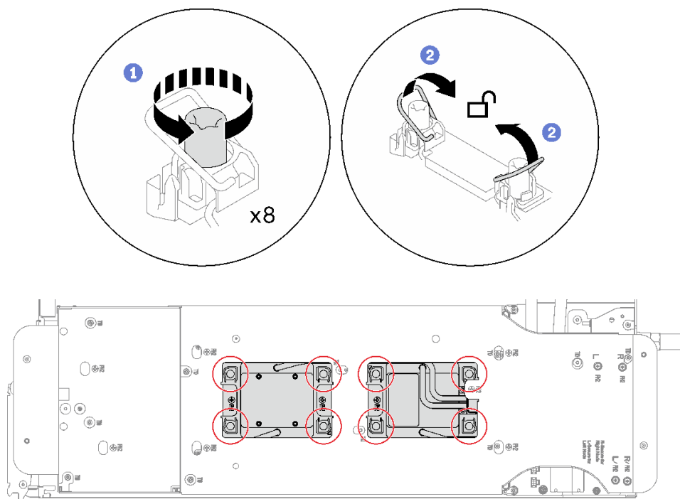
图 212. 松开处理器
