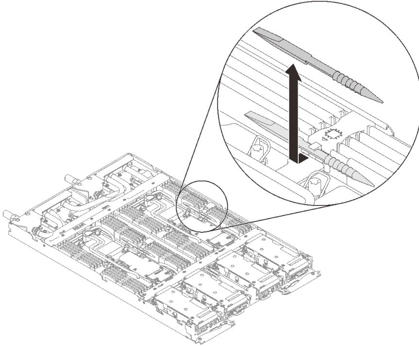
图 135. 卸下内存条工具
