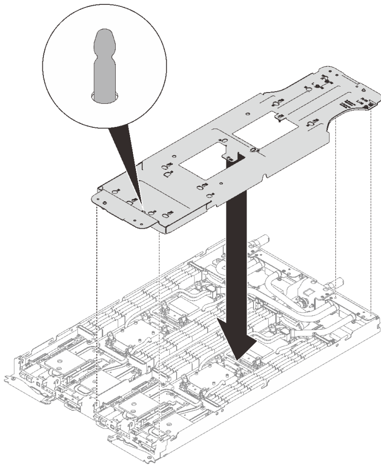
图 192. 安装水循环模块载板
