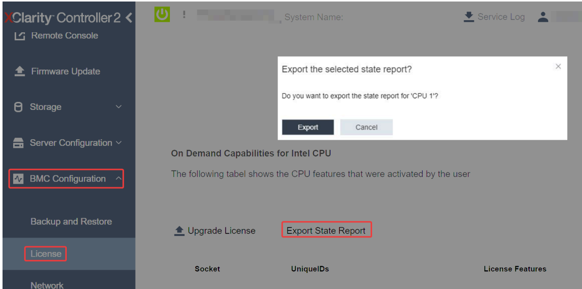
图 247. 通过 XCC Web GUI 导出状态报告
