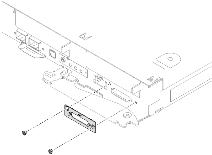
图 122. 安装 KVM 外盖
