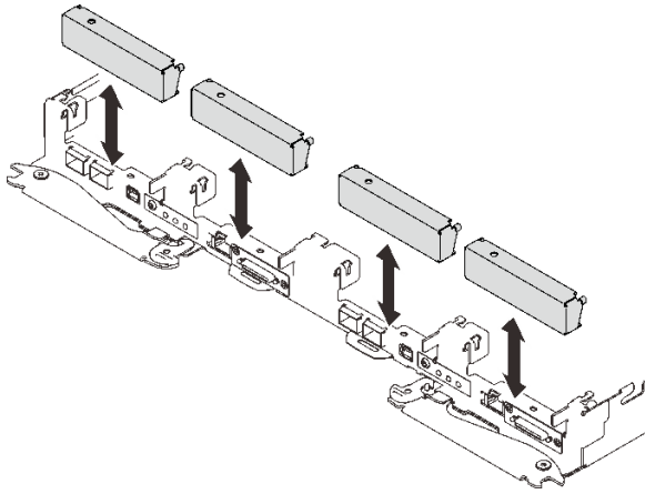
图 169. 安装空挡板填充件
