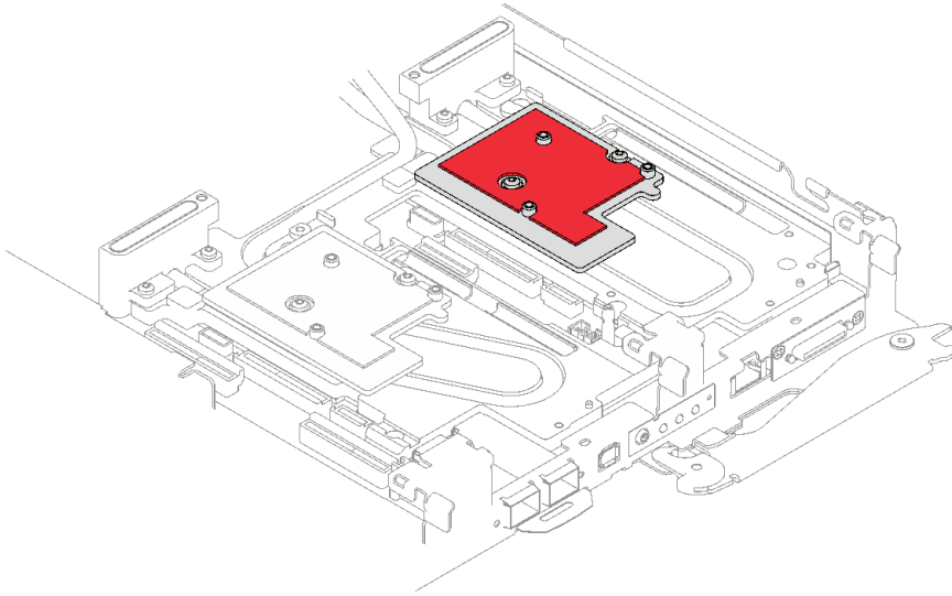
图 187. 适用于 CX-7 NDR 400 的接口板间隙垫
