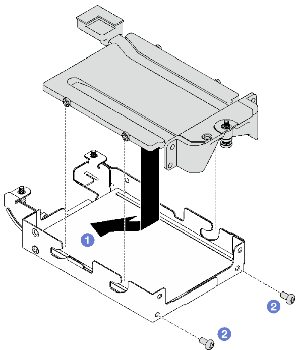
图 111. 安装 E3.S 硬盘导电板
