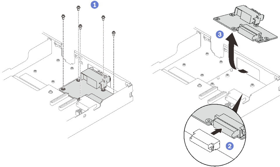
图 196. 卸下配电板
