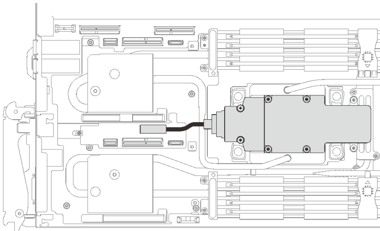
图 130. 安装 M.2 背板组合件线缆
