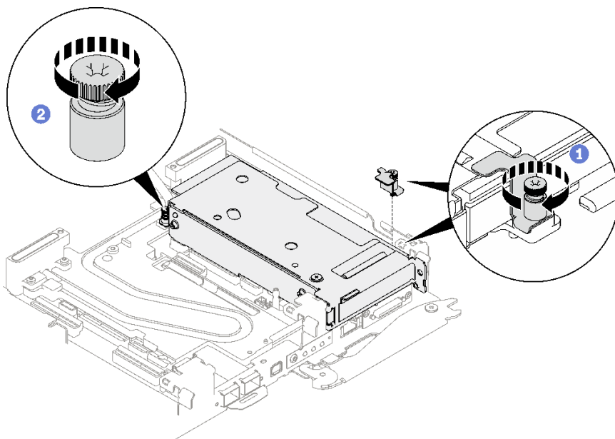
图 161. 安装夹持支架的松不脱螺钉
