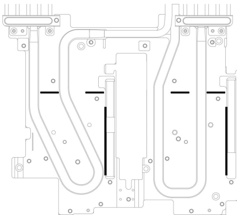
图 117. 水循环模块上的 E3.S 间隙垫对齐标记
