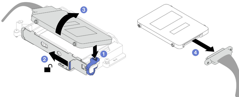
Figura 110. Extracción de la unidad superior (NVMe de 7 mm)
