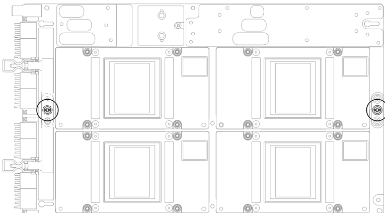
Figura 371. Extracción de los tornillos T15 del conjunto de la placa de la GPU
