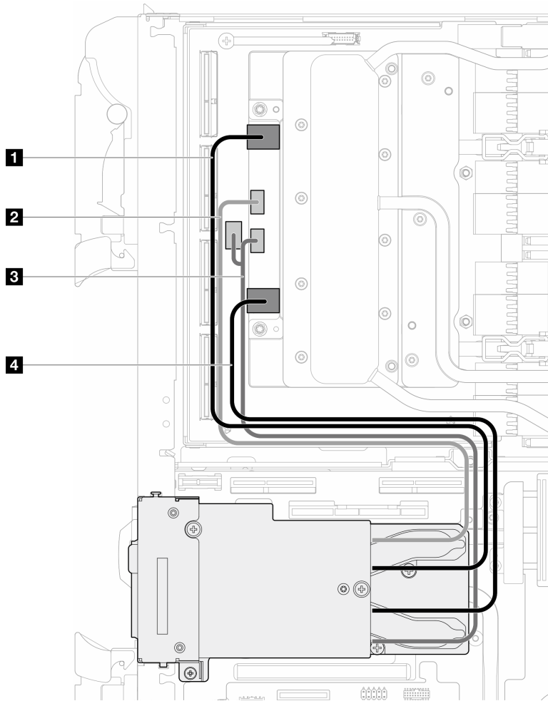
Figura 414. Desconexión de los cables del módulo OSFP de la placa de red
