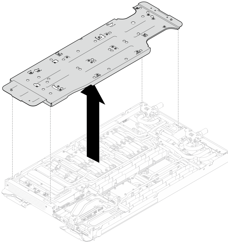
Figura 61. Extracción del transportador del bucle de agua (nodo de la GPU)
