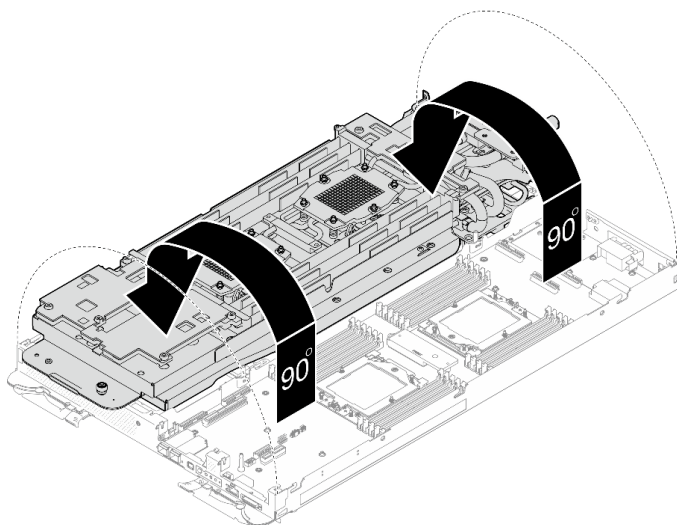
Figura 37. Doblar el bucle de agua
