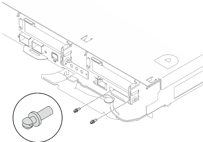
Figura 304. Instalación de los tornillos KVM
