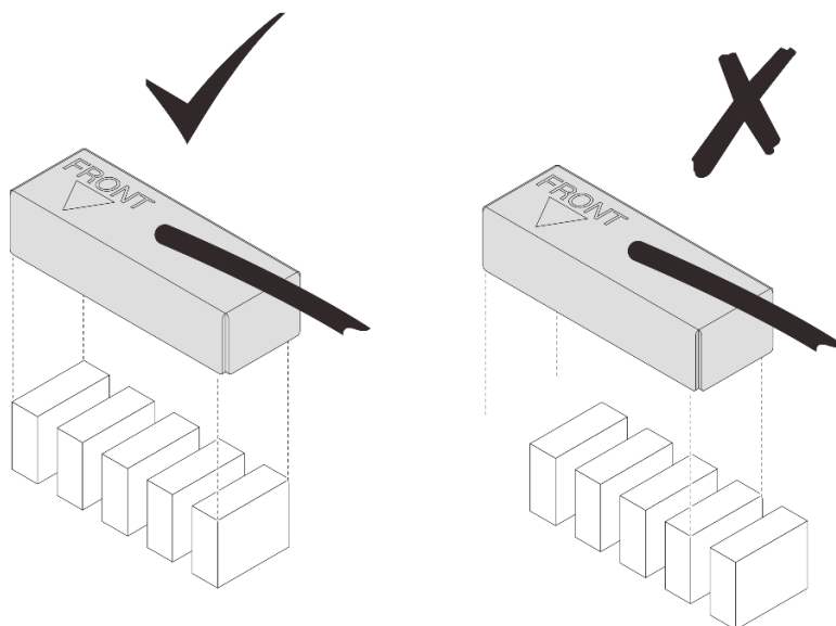
Figura 291. Cubierta de los inductores con el compartimiento protector
