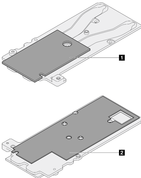
Figura 57. Sustitución de las almohadillas de masilla de la placa de conducción del módulo OSFP
