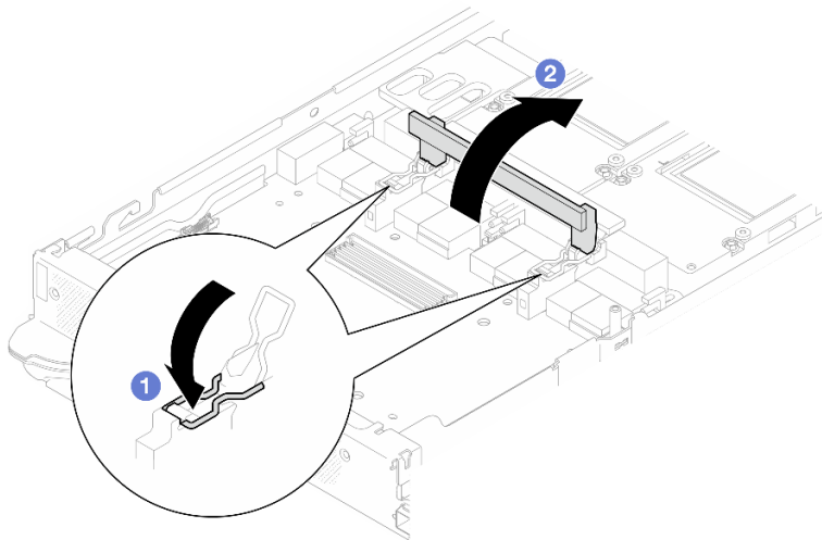
Figura 317. Fijación de la placa del transportador a la placa de la GPU
