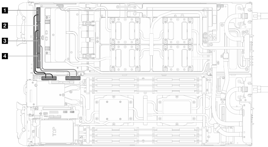
Figura 168. Configuración de un procesador: desconecte todos los cables MCIO
