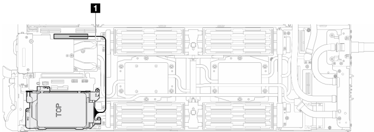
Figura 120. Conexión de los cables del compartimiento de la unidad
