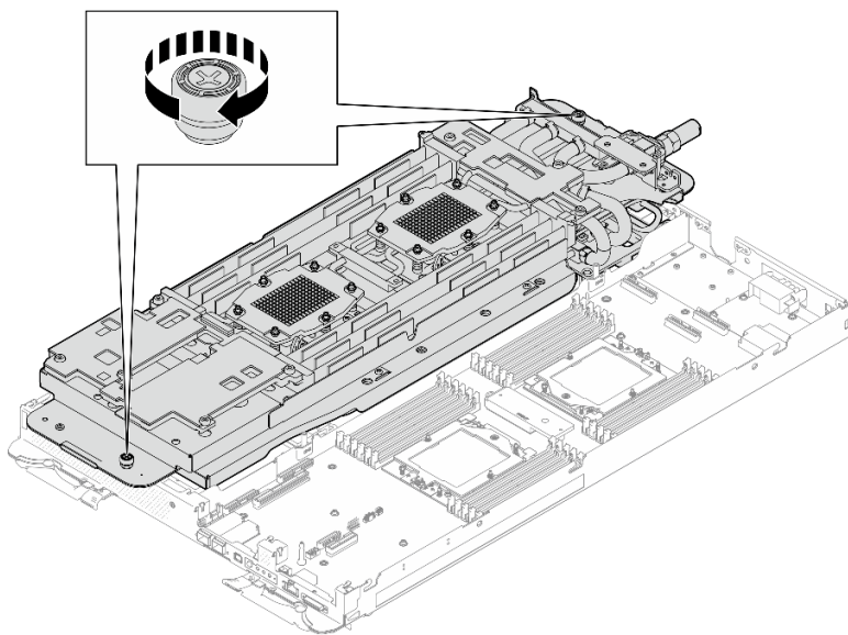
Figura 38. Apriete de los tornillos ajustables cautivos
