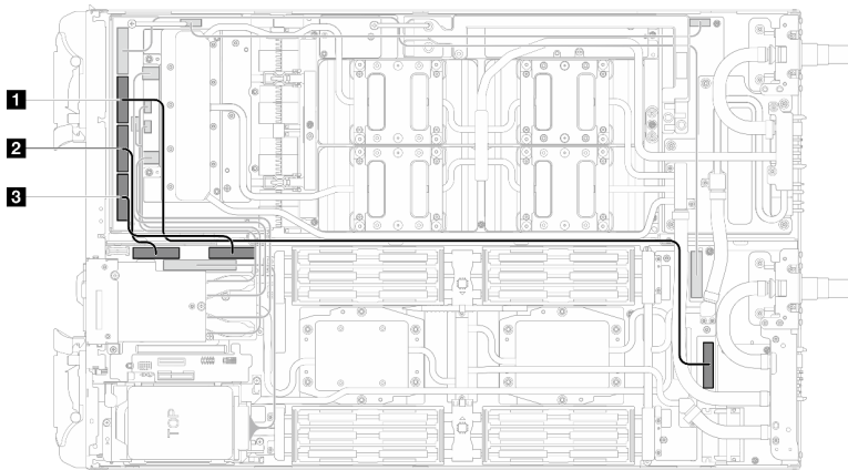
Figura 179. Configuración de dos procesadores - Conexión de los cables MCIO 2, MCIO 3 y MCIO 4 al nodo de la GPU
