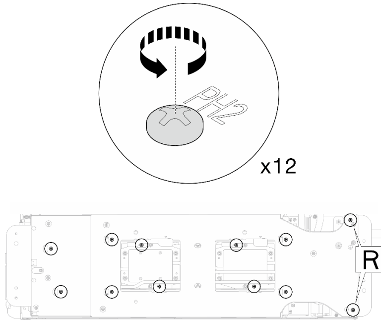
Figura 232. Soltar los tornillos del transportador del bucle de agua
