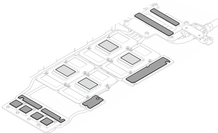
Figura 341. Sustitución de almohadillas de masilla del bucle de agua (nodo de GPU)
