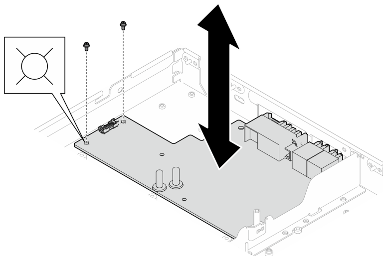
Figura 396. Extracción de los tornillos de la placa de distribución de alimentación de la GPU
