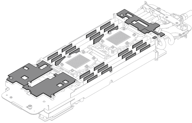
Figura 256. Almohadillas de espacio del bucle de agua (parte inferior)
