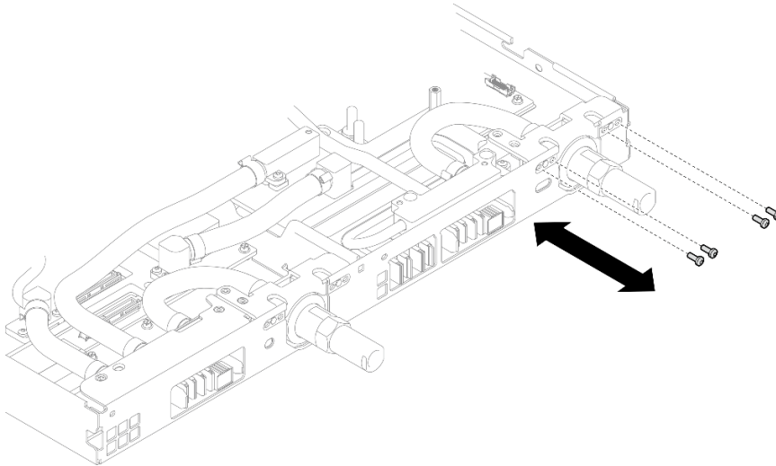
Figura 325. Extracción del tornillo de la conexión rápida (nodo de la GPU)
