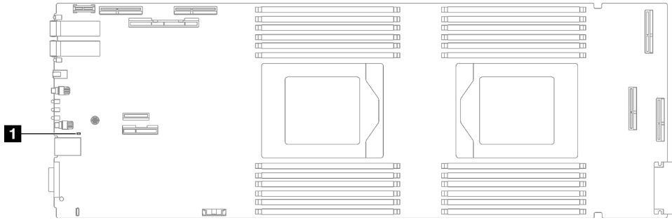
Figura 462. LED de la placa del sistema
