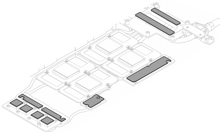
Figura 395. Limpieza de las almohadillas de masilla del bucle de agua
