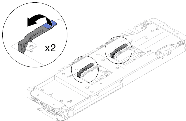
Figura 250. Separe el bucle de agua del procesador
