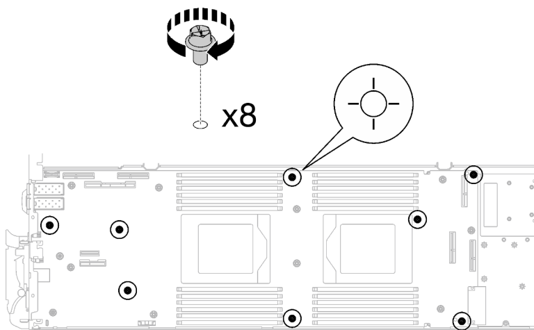
Figura 307. Instalación de los tornillos de la placa del sistema
