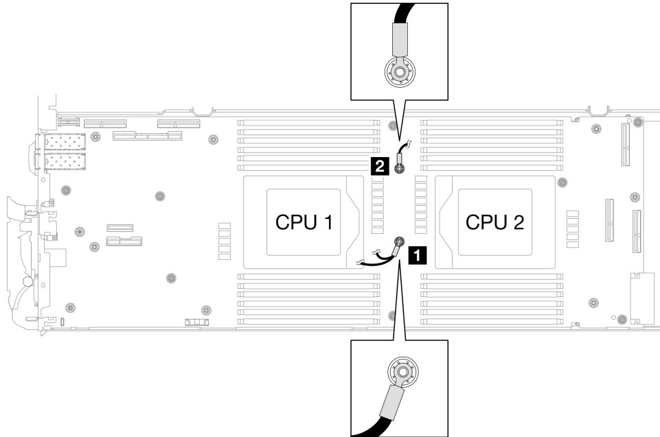
Figura 72. Alineación del cable protector 1/2 y cable protector 3 con los orificios para tornillos
