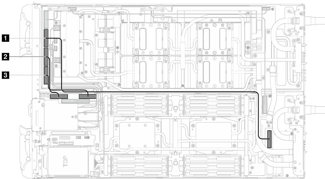
Figura 169. Configuración de dos procesadores - Desconexión de los cables MCIO 2, MCIO 3 y MCIO 4
