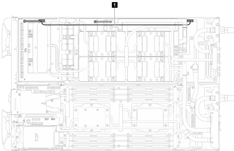
Figura 446. Conexión del cable de alimentación de la placa del transportador
