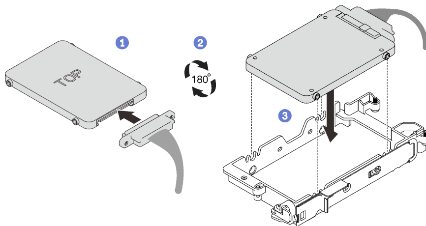
Figura 98. Instalación de la unidad inferior (unidad de 7 mm)
