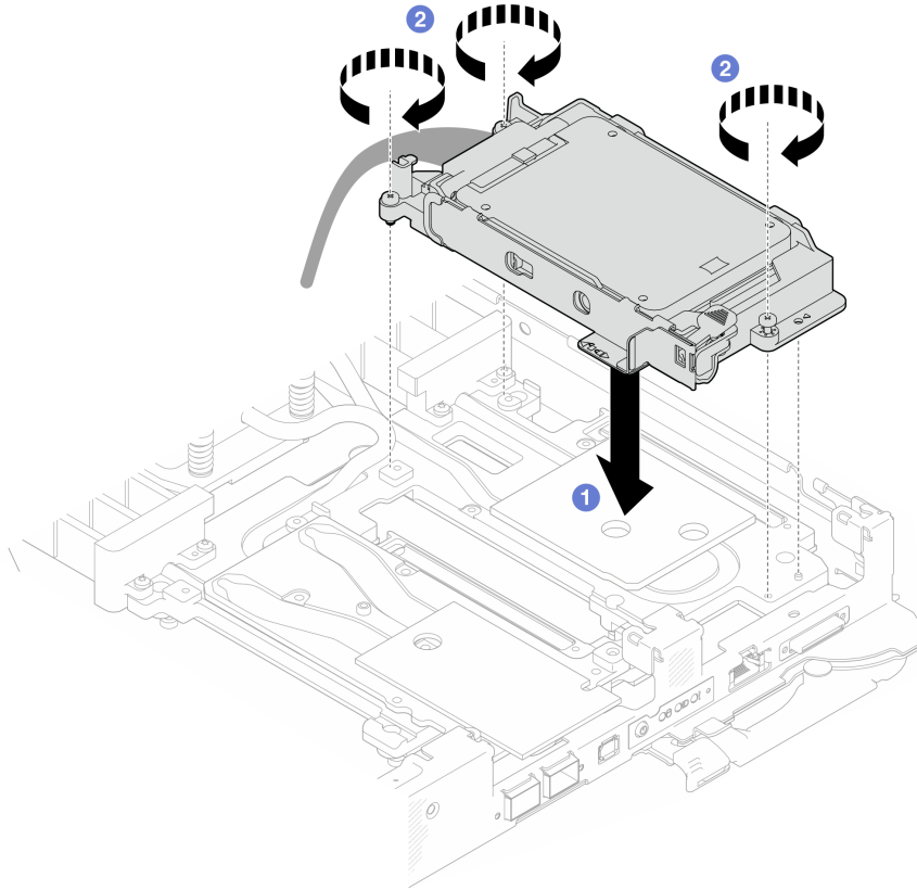
Figura 119. Instalación del conjunto del compartimiento de la unidad NVMe de 7 mm
