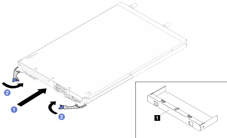
Figura 4. Instalación de la bandeja
