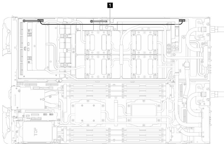
Figura 321. Extracción del cable de alimentación de la placa del transportador
