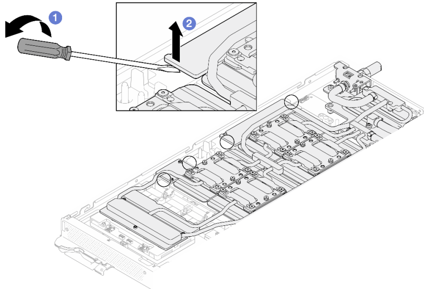
Figura 328. Las placas de conducción MISC delantera y trasera se sueltan ligeramente de la placa de la GPU
