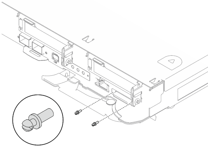
Figura 270. Extracción de tornillos KVM
