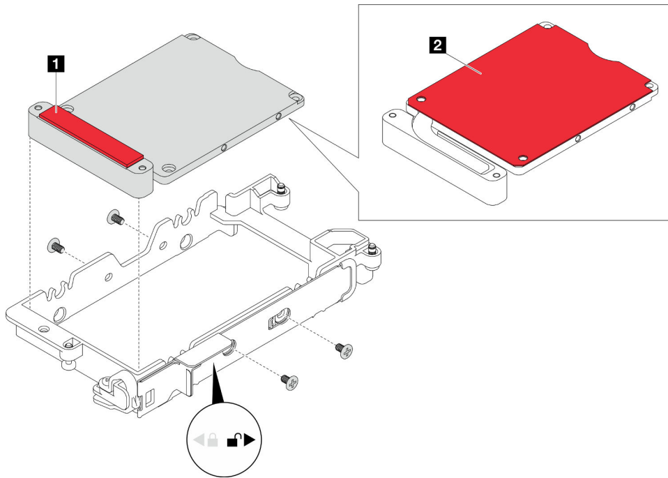
Figura 97. Instalación de la placa de conducción
