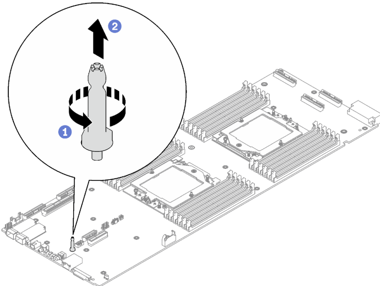
Figura 274. Extracción de la patilla guía
