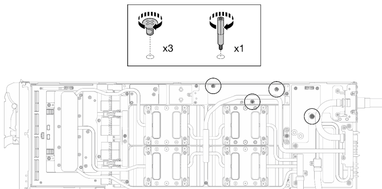
Figura 444. Instalación de los tornillos hexagonal y PH1 del bucle de agua (nodo de la GPU)
