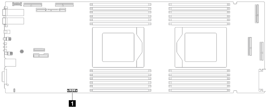
Figura 79. Ubicación de batería CMOS
