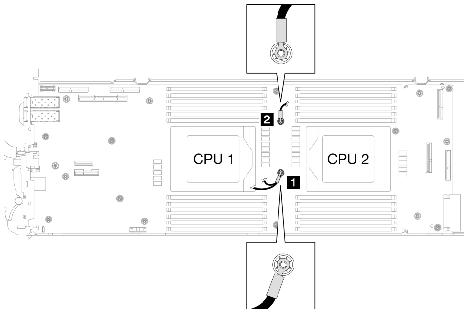
Figura 279. Alineación del cable protector 1/2 y cable protector 3 con los orificios para tornillos
