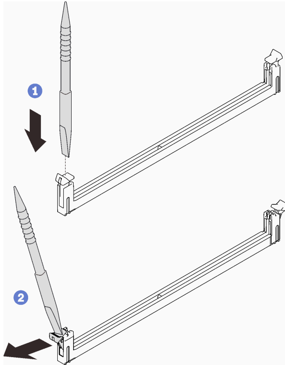
Figura 162. Cómo presionar los clips de sujeción en el conector del módulo de memoria
