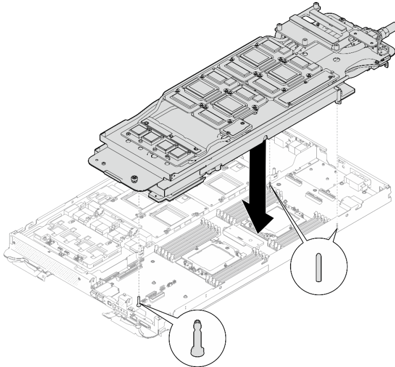
Figura 49. Instalación del transportador del bucle de agua
