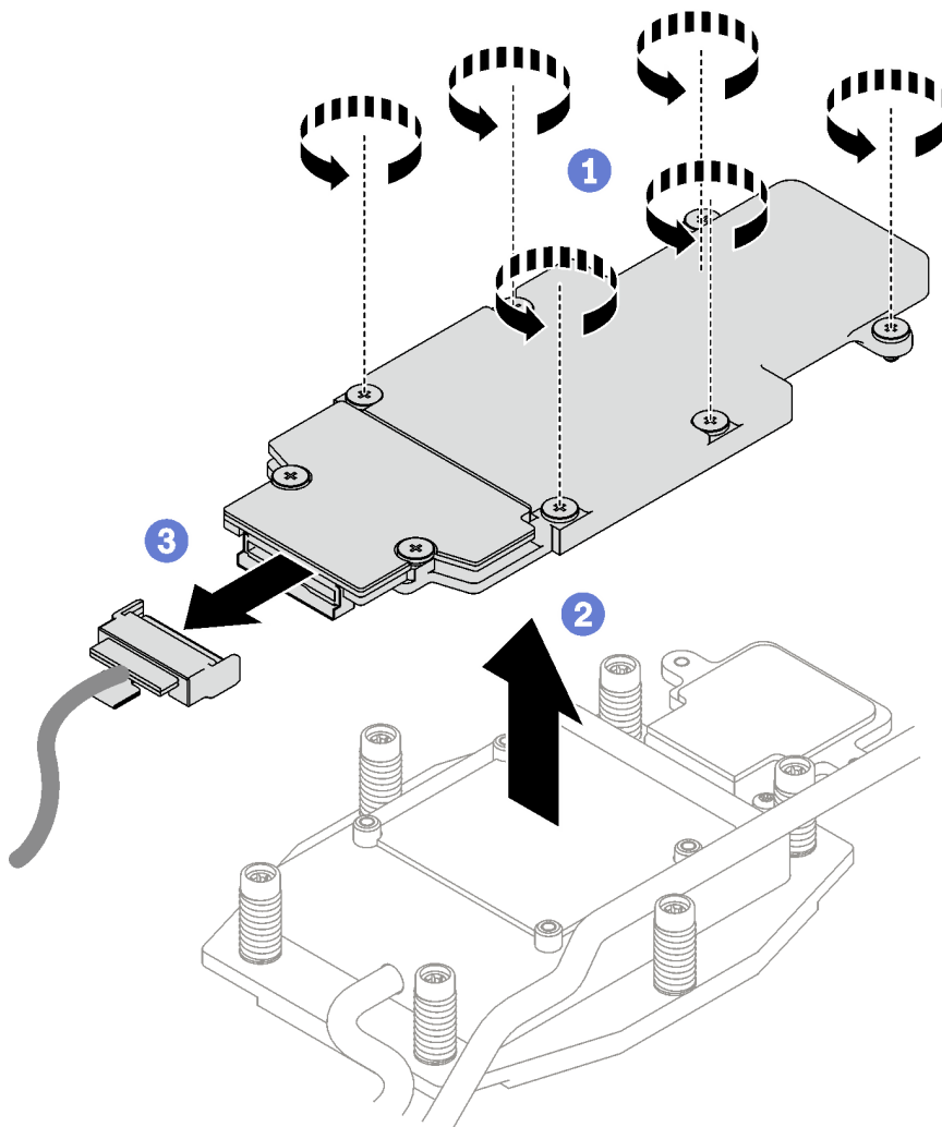
Figura 143. Extracción del conjunto de placas posteriores de M.2
