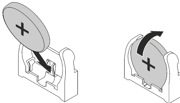
Figura 82. Instalación de la batería CMOS
