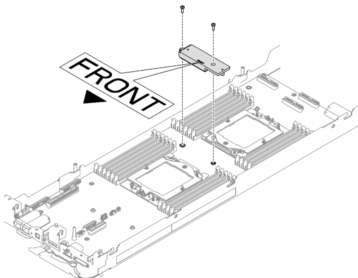
Figura 306. Instalación de la placa de conducción del VR
