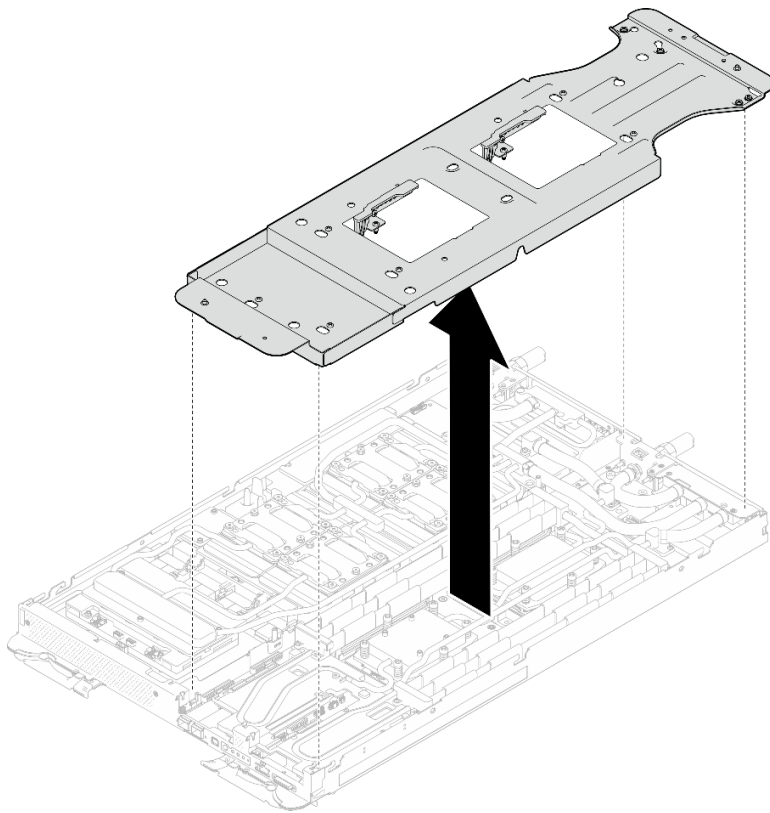
Figura 52. Extracción del transportador del bucle de agua (nodo de cálculo)
