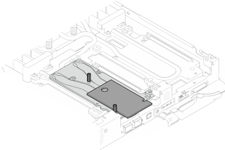
Figura 174. Sustitución de la almohadilla de masilla en el módulo OSFP
