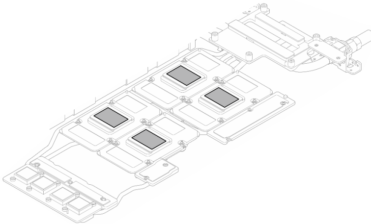
Figura 24. Limpieza del PCM de todas las GPU
