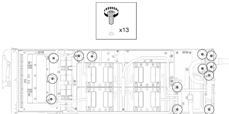
Figura 65. Instalación de los tornillos Torx T10 del bucle de agua (nodo de la GPU)
