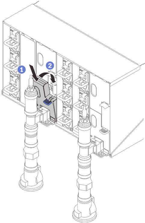
Figura 468. Instalación del protector EMC
