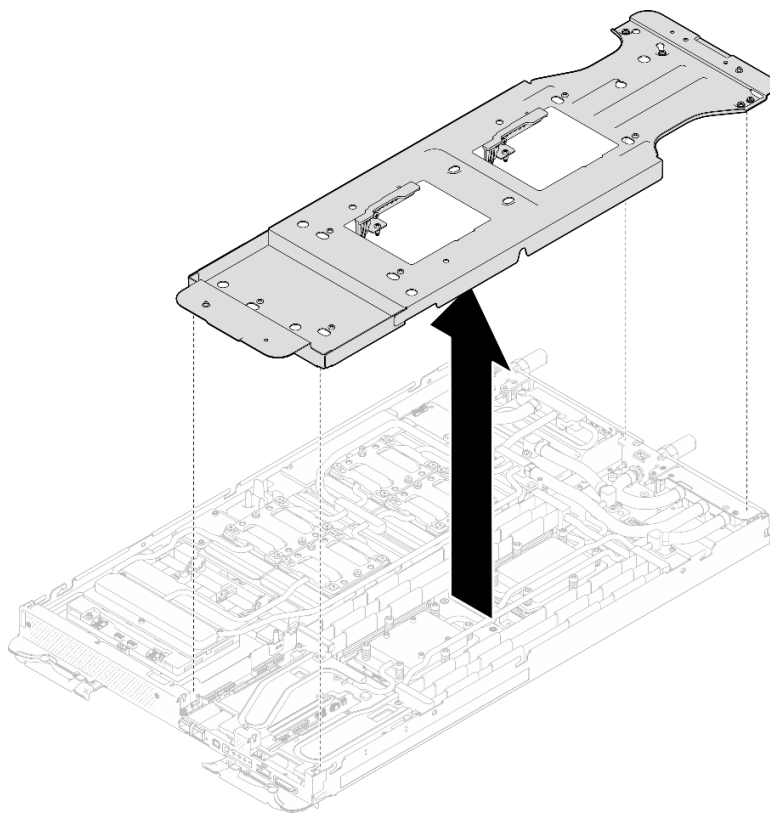
Figura 233. Extracción del transportador del bucle de agua (nodo de cálculo)
