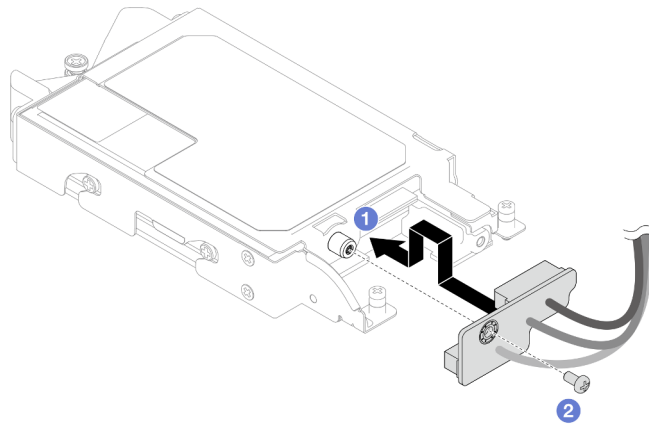
Figura 135. Instalación de la placa posterior con cable de la unidad E3.s
