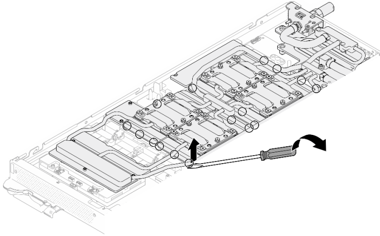
Figura 330. Liberación de la placa de frío de la GPU desde la GPU
