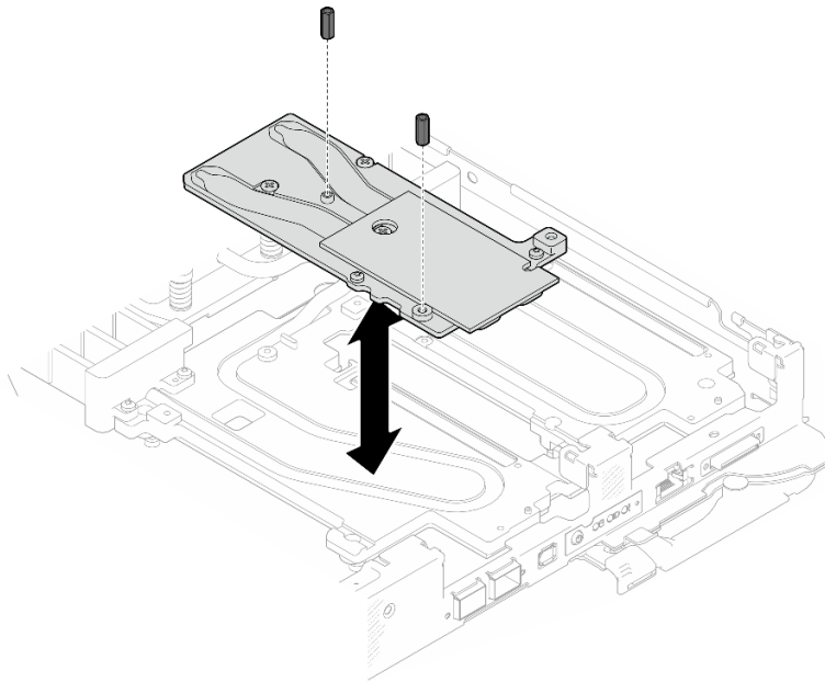
Figura 241. Extracción de los tornillos hexagonales de la placa de conducción de Módulo OSFP
