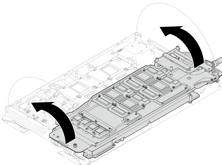
Figura 437. Despliegado del bucle de agua en el nodo de la GPU
