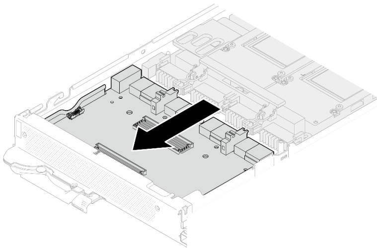
Figura 355. Desconexión de la placa del transportador de la placa de la GPU
