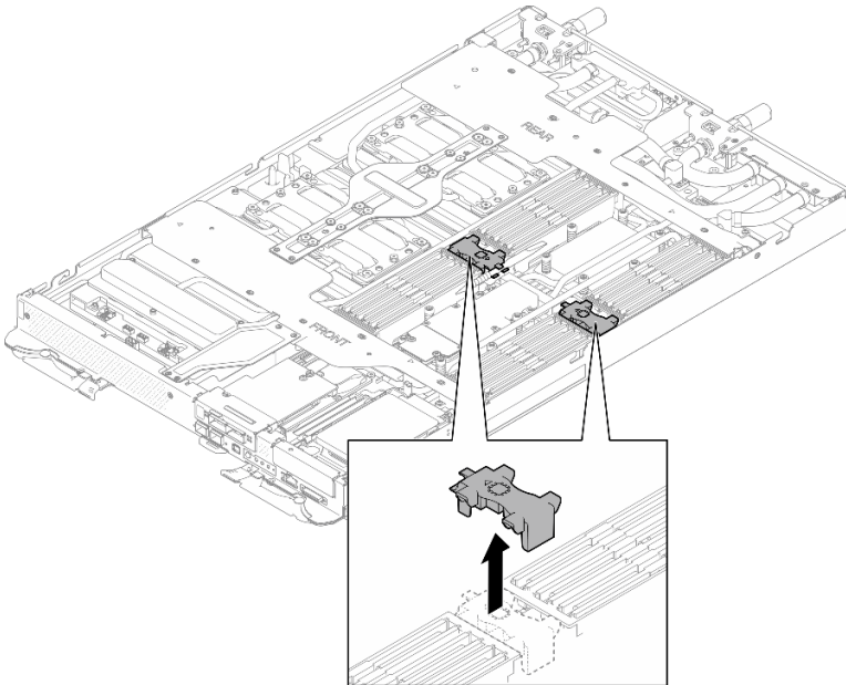
Figura 84. Extracción de la guía de DIMM
