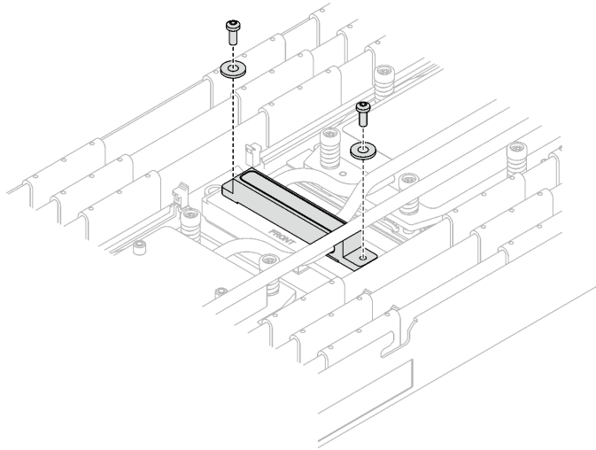
Figura 54. Tornillos de la placa de frío del VR con arandela
