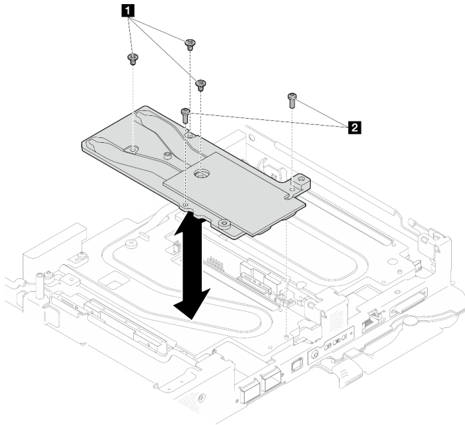
Figura 268. Instalación de la placa de conducción del Módulo OSFP
