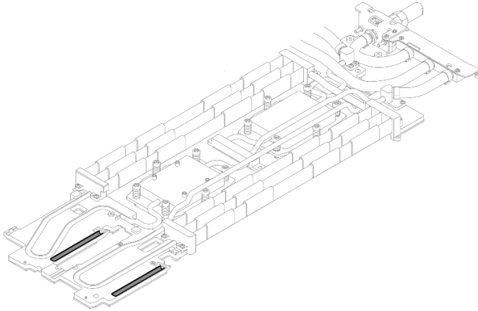
Figura 45. Almohadillas de espacio de la parte superior del bucle de agua (lado del nodo de cálculo)
