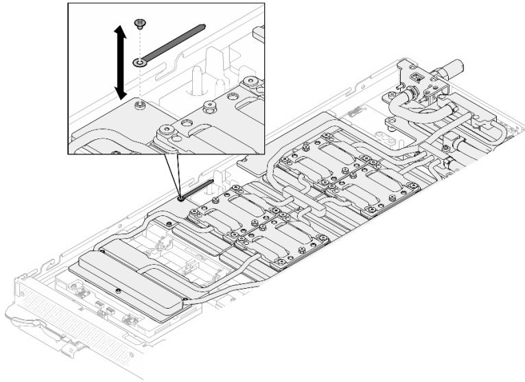
Figura 351. Instalación de la brida de cables
