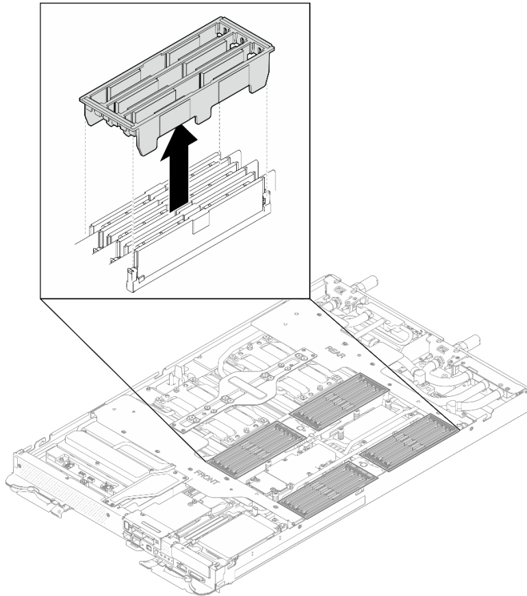
Figura 161. Extracción de la cubierta DIMM
