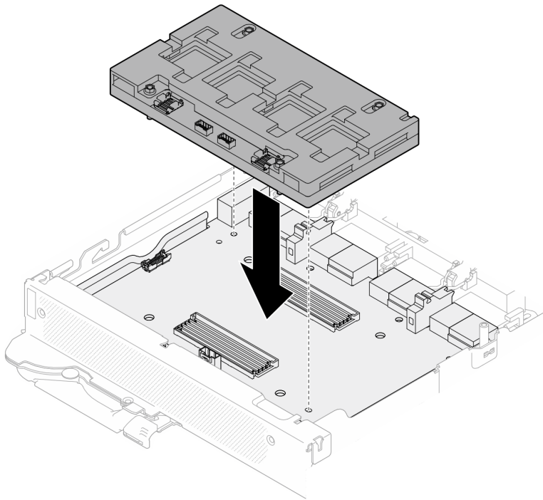
Figura 432. Instalación de la placa de red
