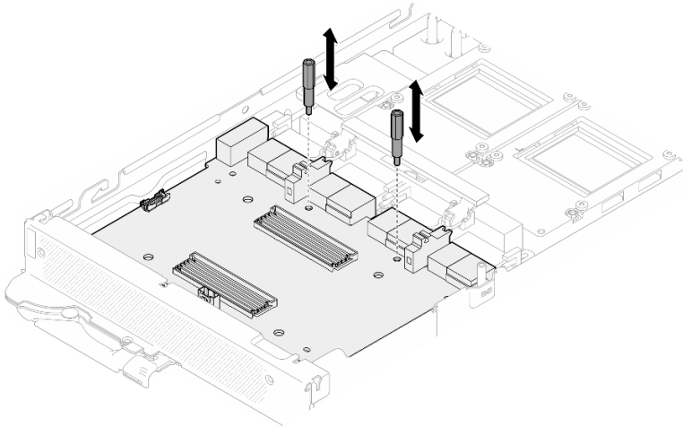
Figura 353. Extracción de los aisladores de la placa del transportador
