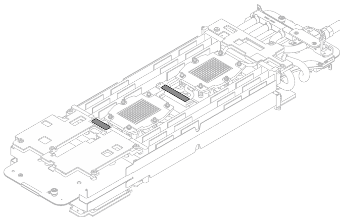
Figura 229. Almohadillas de masilla en el bucle de agua
