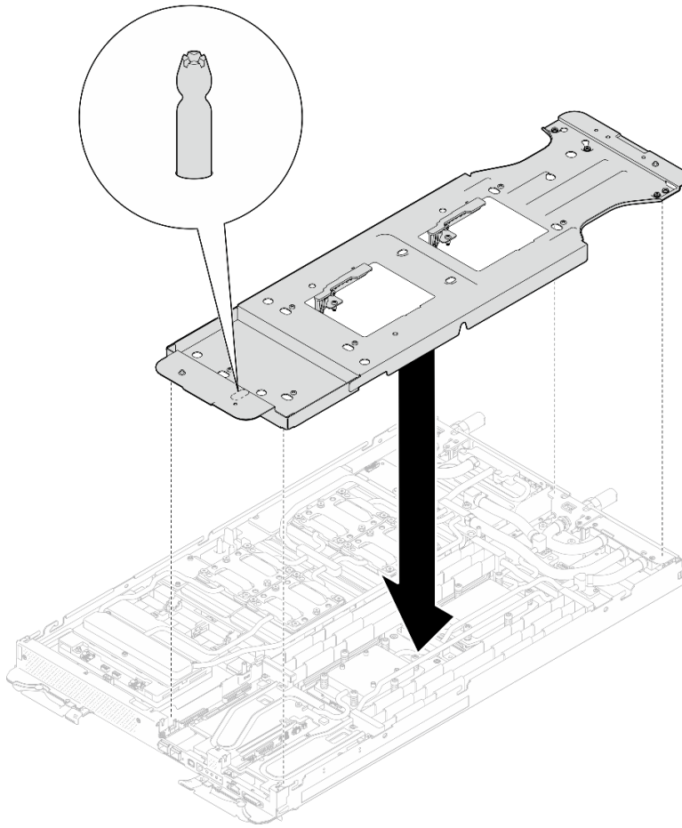
Figura 189. Instalación del transportador del bucle de agua (nodo de cálculo)
