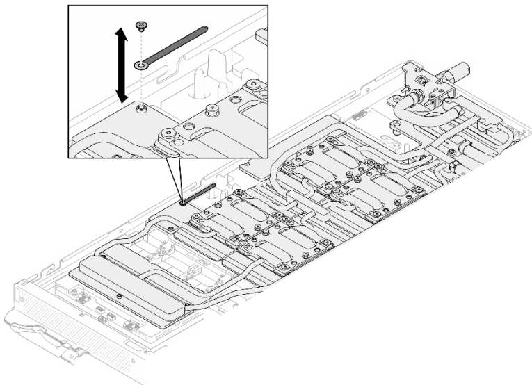
Figura 382. Extracción de la brida de cables
