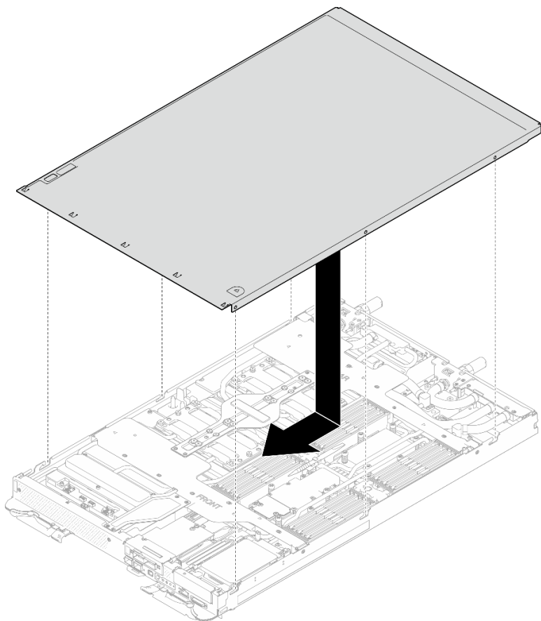
Figura 6. Instalación de la cubierta de la bandeja
