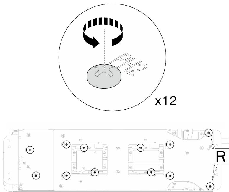
Figura 249. Instalación de los tornillos del transportador del bucle de agua (nodo de cálculo)
