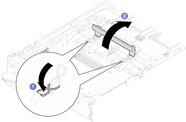
Figura 365. Fijación de la placa del transportador a la placa de la GPU
