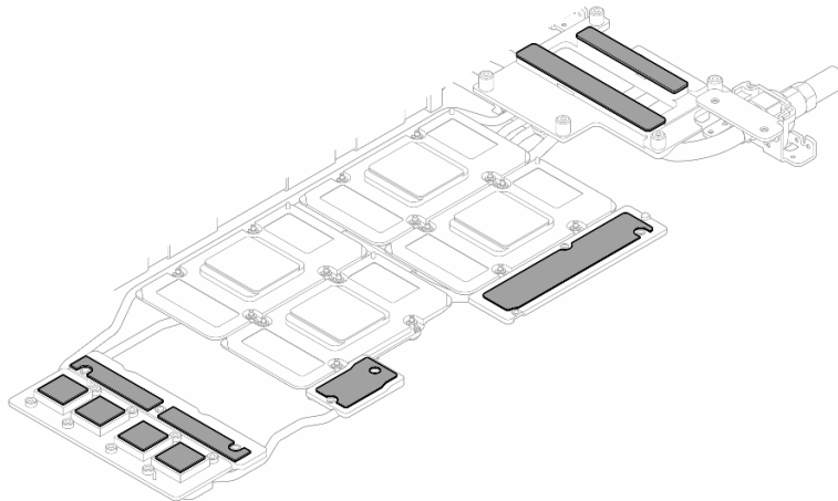
Figura 335. Limpieza de las almohadillas de masilla del bucle de agua
