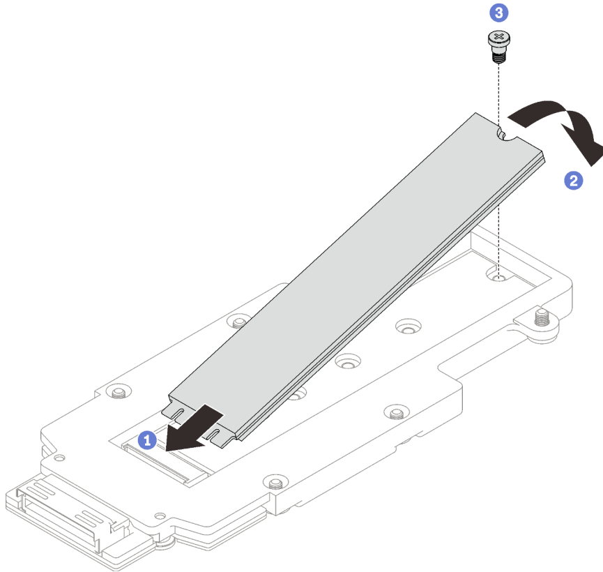
Figura 146. Instalación de la unidad M.2
