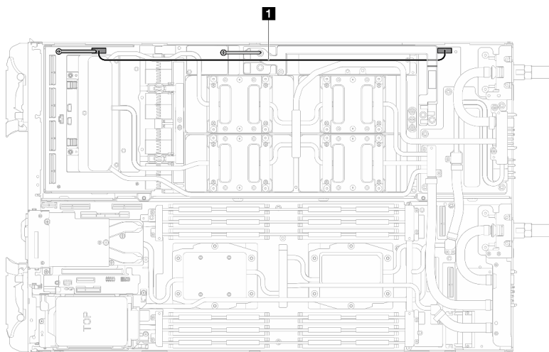
Figura 415. Extracción del cable de alimentación de la placa del transportador
