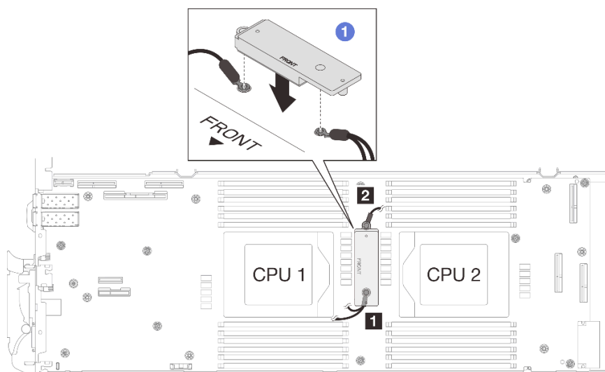
Figura 280. Alineación de la placa de conducción de VR, cables protectores y orificios para los tornillos de la placa del sistema
