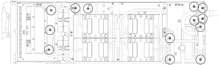
Figura 324. Extracción de los tornillos Torx T10 del bucle de agua (nodo de la GPU)
