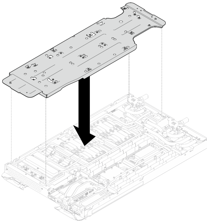
Figura 331. Instalación del transportador del bucle de agua (nodo de la GPU)
