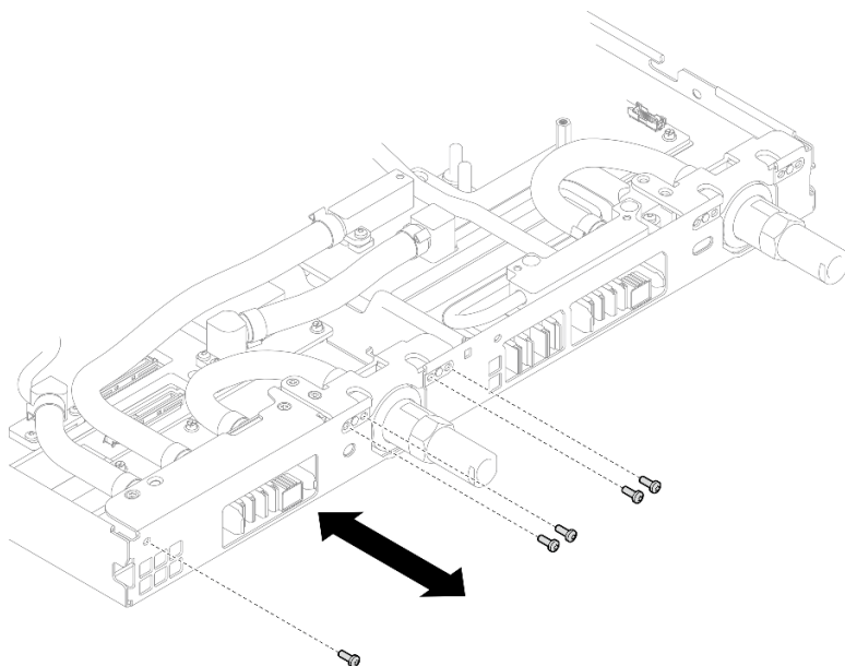
Figura 266. Instalación del tornillo de la conexión rápida (nodo de cálculo)
