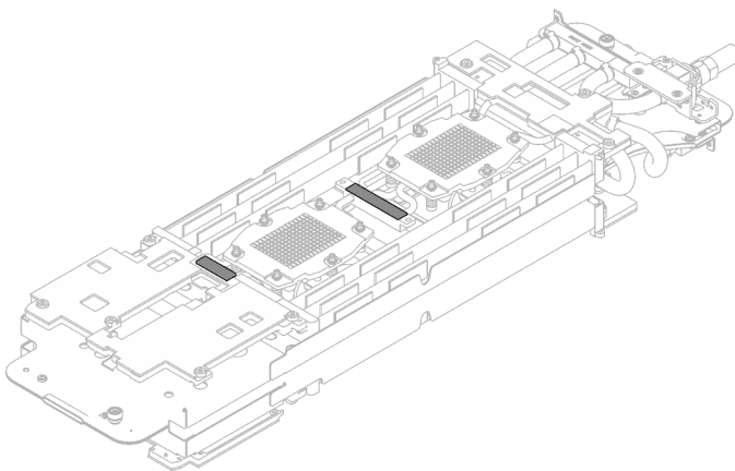
Figura 258. Almohadillas de masilla en el bucle de agua
