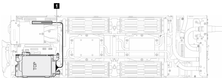
Figura 166. Desconexión del cable de la unidad
