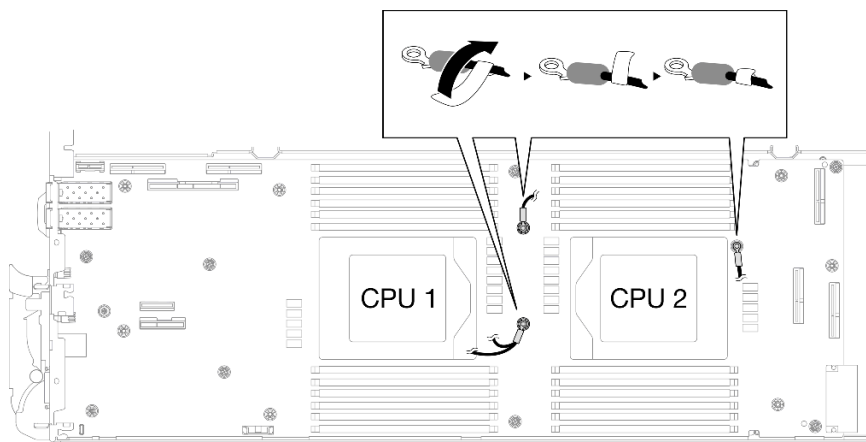
Figura 285. Etiqueta alrededor del cable protector
