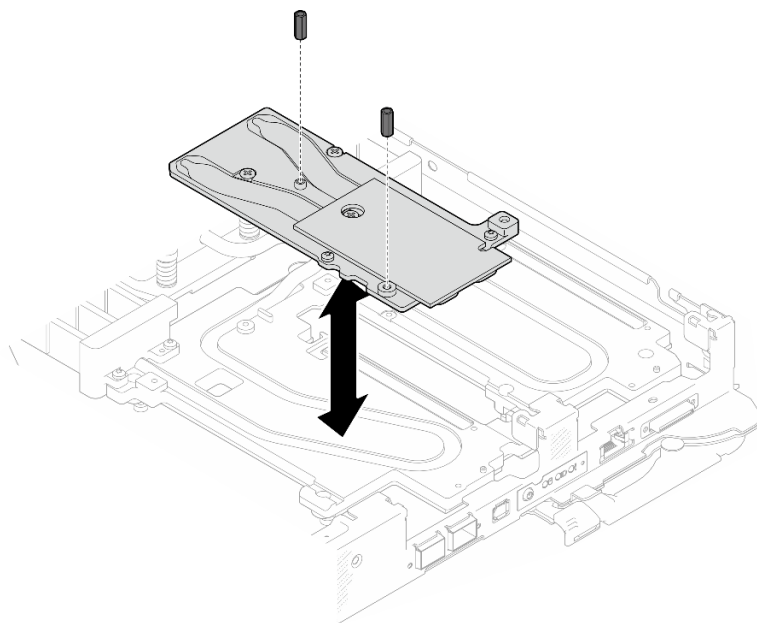
Figura 240. Instalación de los tornillos hexagonales de la placa de conducción de Módulo OSFP
