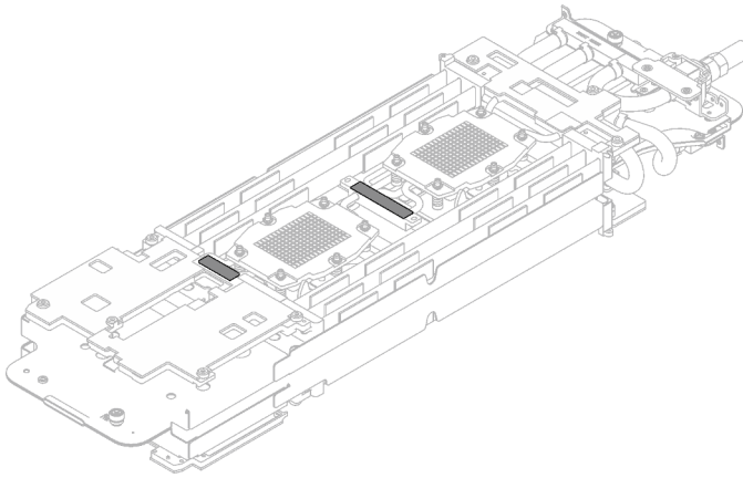
Figura 198. Almohadillas de masilla en el bucle de agua
