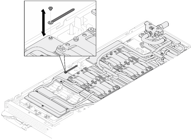
Figura 322. Extracción de la brida de cables
