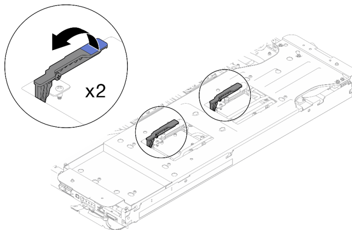
Figura 191. Separe el bucle de agua del procesador
