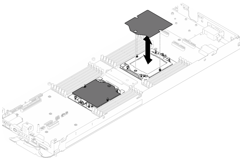
Figura 252. Extracción de la película protectora del zócalo del procesador
