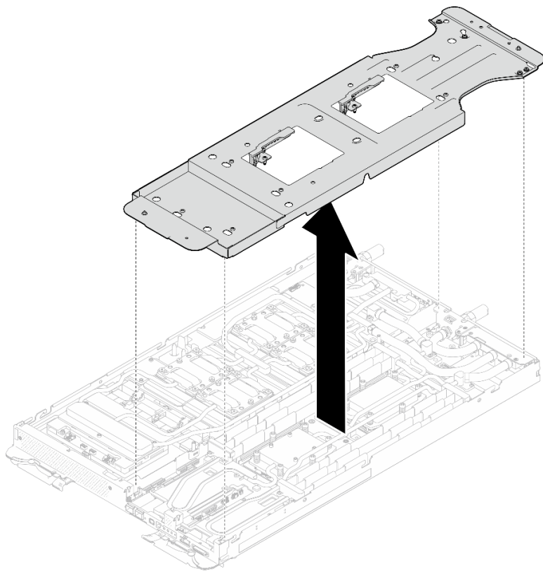
Figura 262. Extracción del transportador del bucle de agua (nodo de cálculo)
