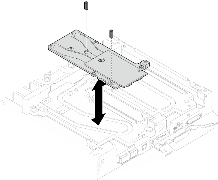
Figura 182. Extracción de los tornillos hexagonales de la placa de conducción de Módulo OSFP
