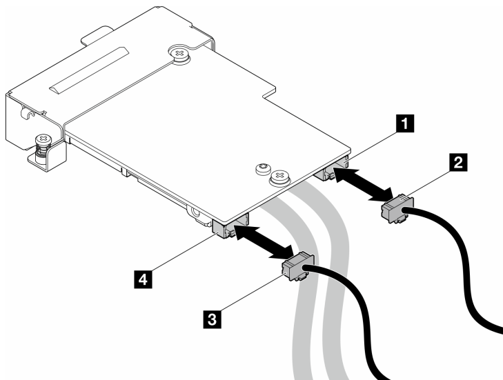
Figura 173. Extracción de los cables de alimentación del módulo OSFP
