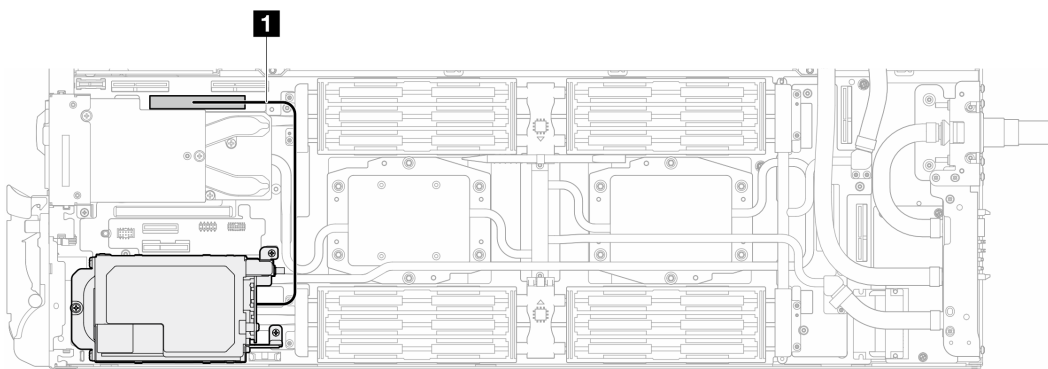
Figura 141. Disposición de los cables de la unidad E3.s
