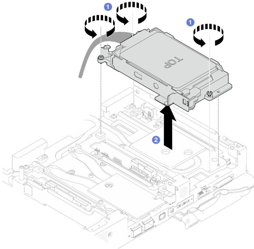
Figura 89. Extracción de dos conjuntos de compartimento de la unidad de 7 mm
