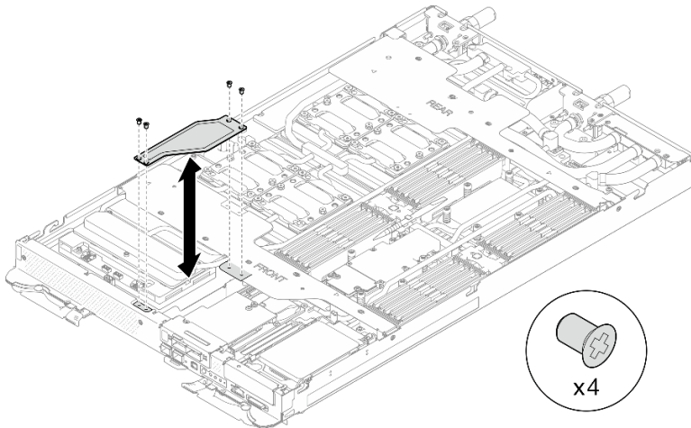
Figura 7. Extracción de la cubierta de cables frontal
