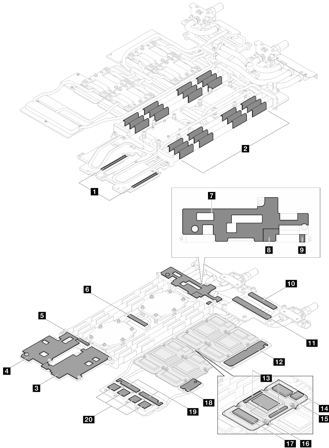
Figura 2. Bucle de agua y nodo de la GPU - Identificación y ubicación de la almohadilla de espacio y la almohadilla de masilla
