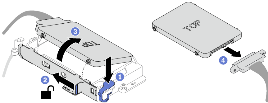
Figura 92. Extracción de la unidad superior
