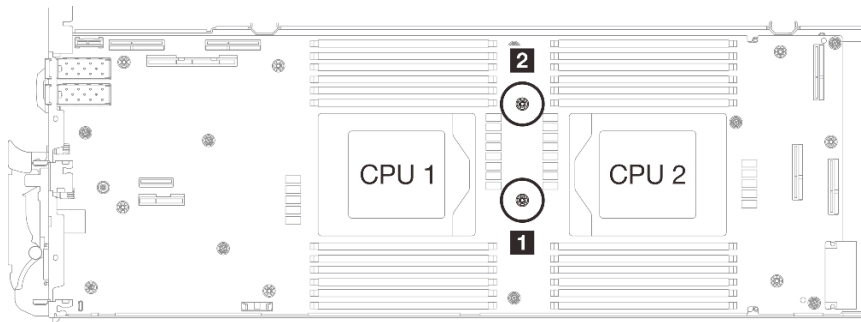
Figura 278. Ubicación de los orificios de tornillo del cable protector 1/2 y 3
