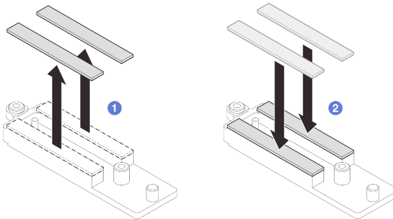
Figura 275. Sustitución de las almohadillas de masilla de la placa de conducción de VR
