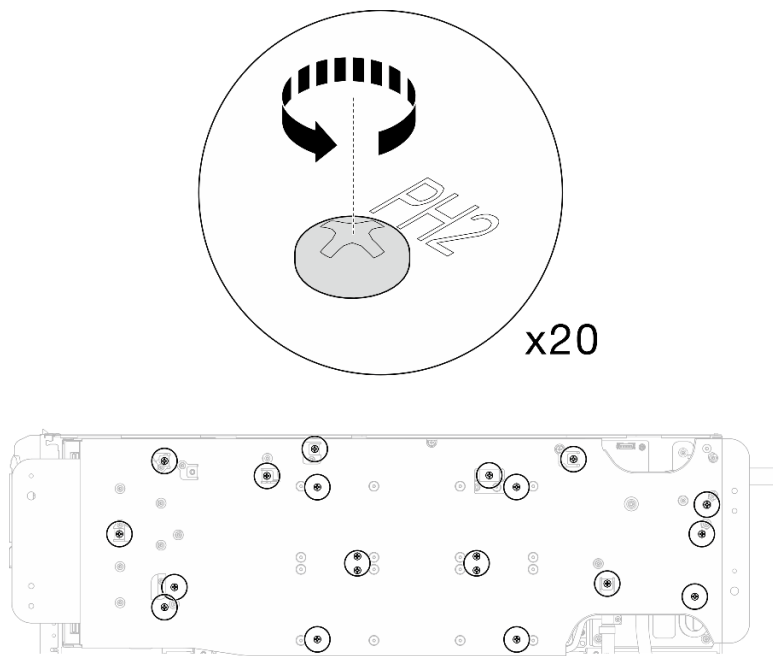
Figura 438. Instalación de los tornillos y tornillos de conexión rápida del bucle de agua (nodo de la GPU)
