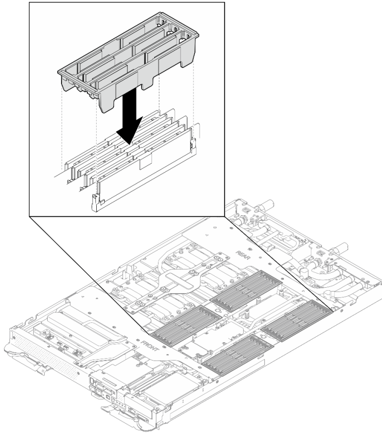
Figura 157. Instalación de la cubierta DIMM
