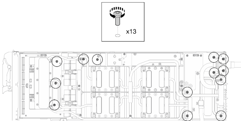
Figura 14. Extracción de los tornillos Torx T10 del bucle de agua (nodo de la GPU)
