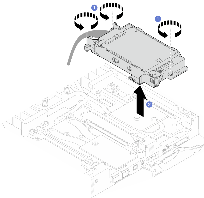
Figura 108. Extracción del conjunto de compartimiento de la unidad NVMe de 7 mm
