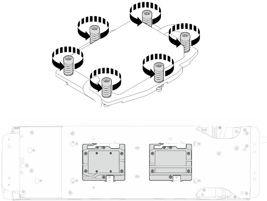
Figura 188. Extracción de la placa de frío del procesador
