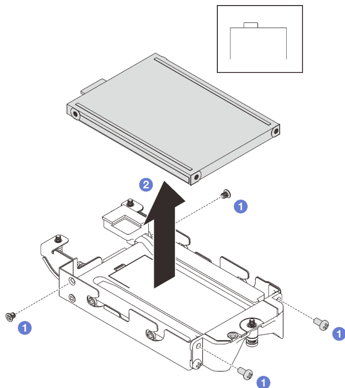
Figura 127. Extracción de la unidad E3.s inferior
