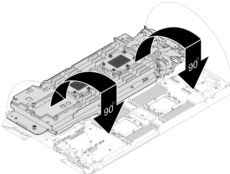
Figura 231. Instalación del bucle de agua
