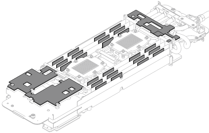
Figura 196. Almohadillas de espacio del bucle de agua (parte inferior)
