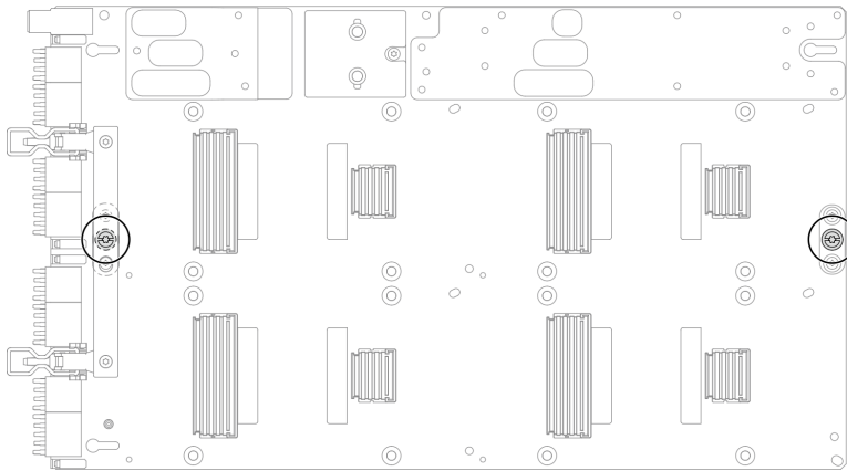
Figura 363. Instalación de los tornillos T15 en la placa de la GPU
