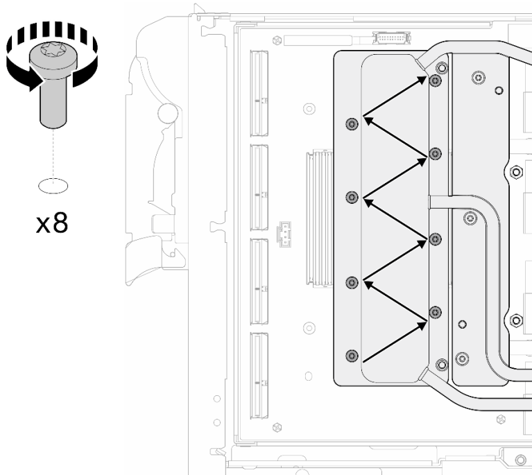
Figura 386. Extracción del tornillo de la tarjeta de red
