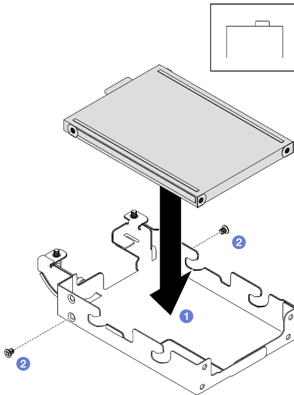
Figura 130. Instalación de la unidad E3.s superior
