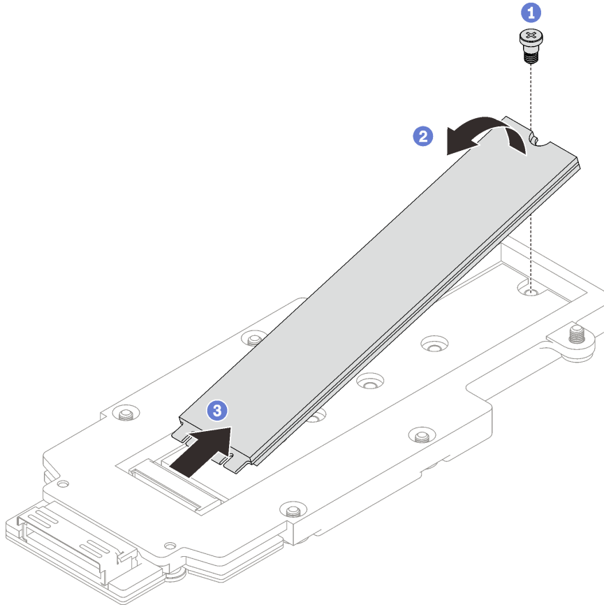
Figura 145. Extracción de la unidad M.2
