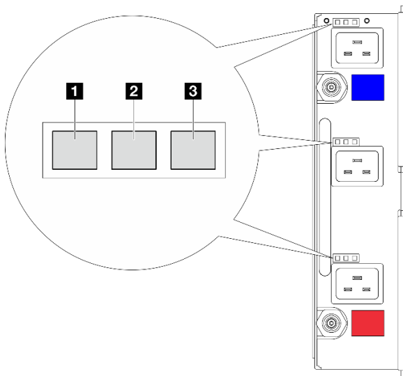
Figura 460. LED del suministro de alimentación de DWC
