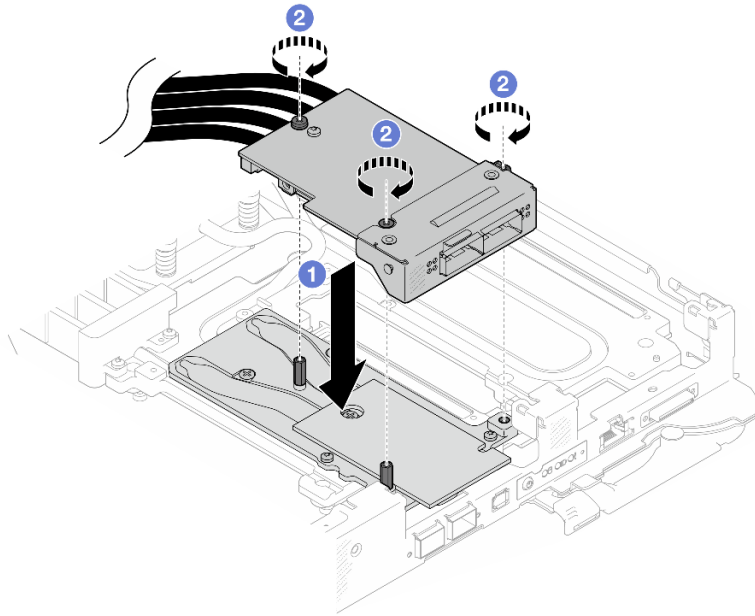
Figura 176. Instalación de la Módulo OSFP
