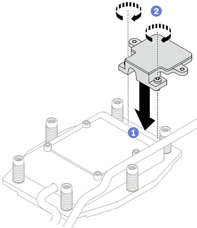
Figura 148. Instalación de la placa de frío de la placa posterior de M.2
