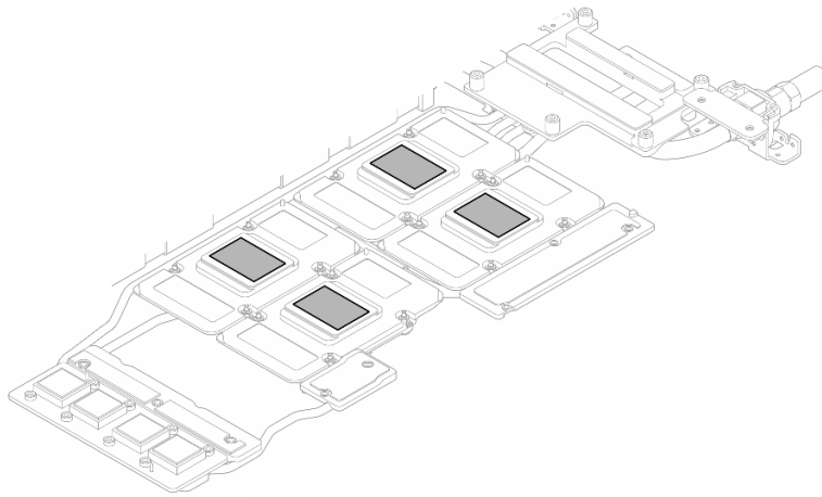
Figura 334. Limpieza del PCM de todas las GPU
