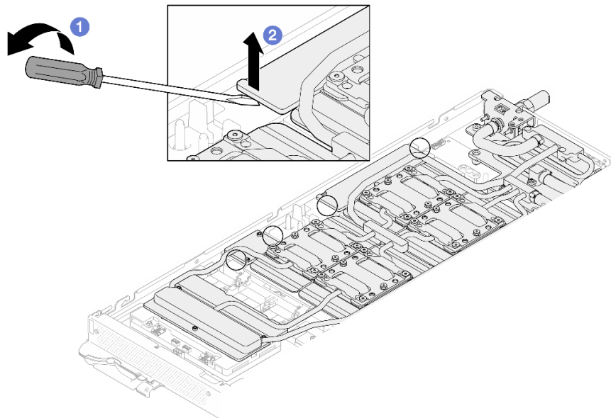
Figura 18. Las placas de conducción MISC delantera y trasera se sueltan ligeramente de la placa de la GPU
