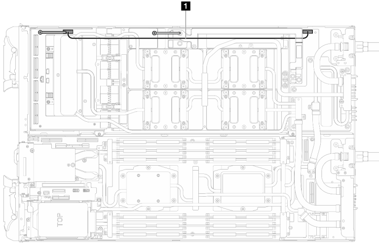
Figura 11. Extracción del cable de alimentación de la placa del transportador
