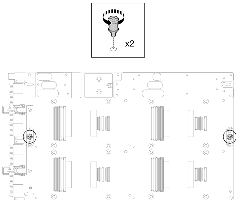
Figura 357. Extracción de los tornillos T15 de la placa de la GPU
