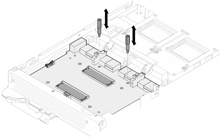
Figura 313. Extracción de los aisladores de la placa del transportador
