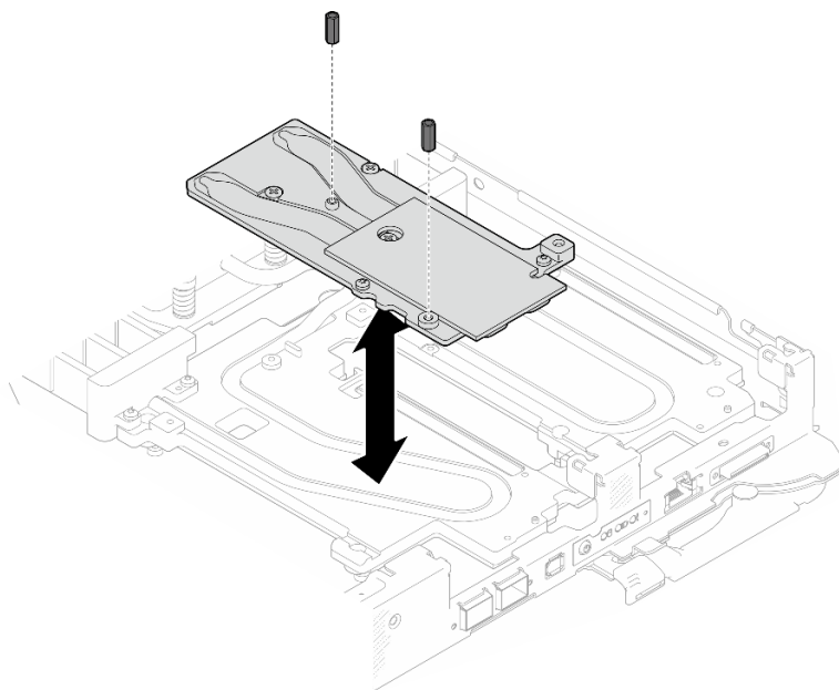
Figura 269. Instalación de los tornillos hexagonales de la placa de conducción de Módulo OSFP
