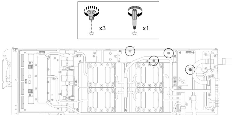
Figura 66. Instalación de los tornillos hexagonal y PH1 del bucle de agua (nodo de la GPU)
