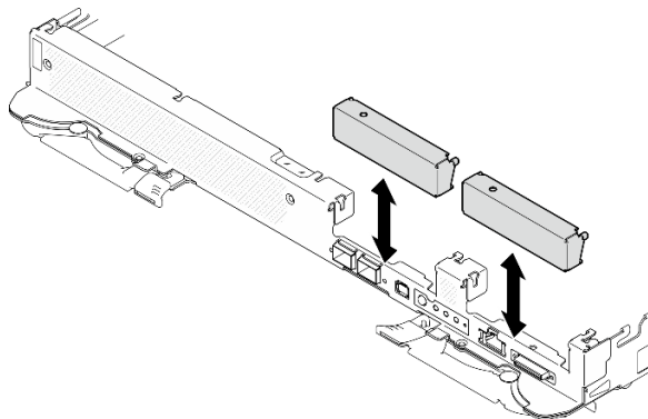
Figura 109. Extracción del relleno vacío del marco biselado
