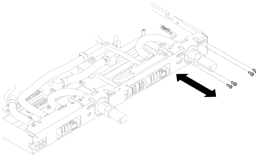
Figura 15. Extracción del tornillo de la conexión rápida (nodo de la GPU)
