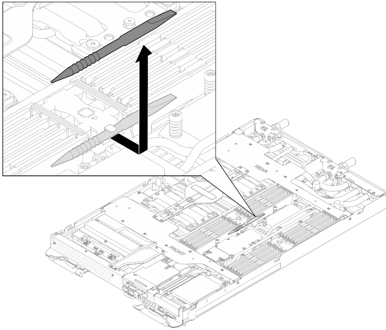
Figura 153. Extracción de la herramienta del módulo de memoria
