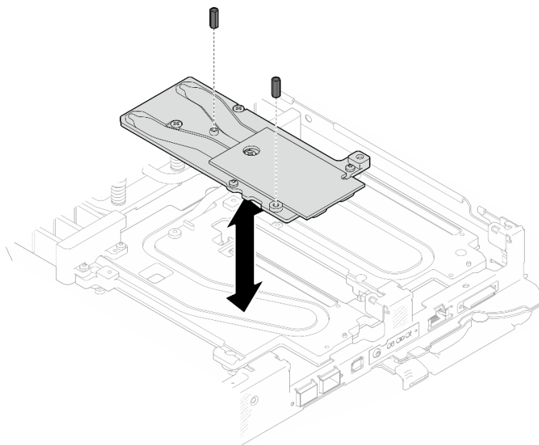
Figura 209. Instalación de los tornillos hexagonales de la placa de conducción de Módulo OSFP
