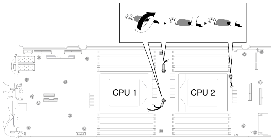
Figura 302. Etiqueta alrededor del cable protector
