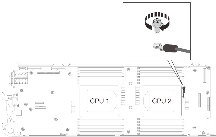
Figura 284. Instalación del cable protector 4
