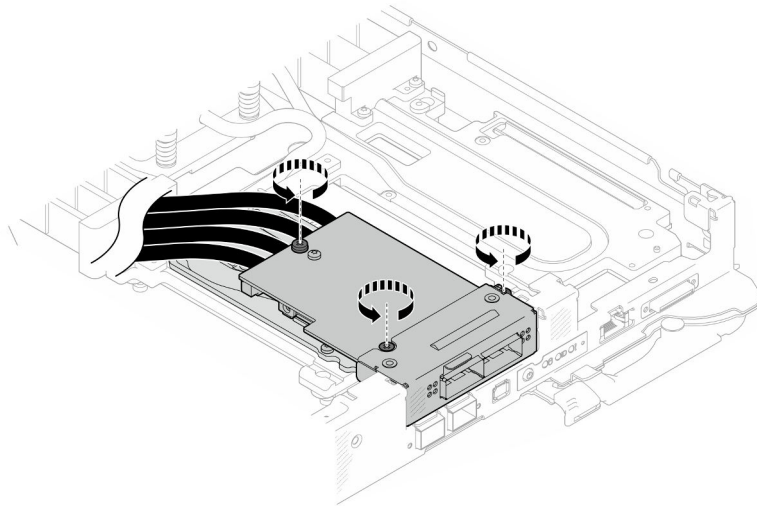
Figura 171. Extracción del Módulo OSFP
