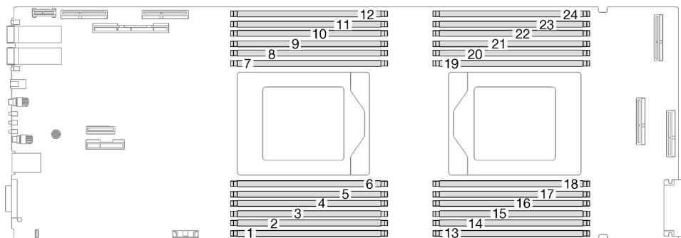
Figura 159. Ubicación del conector del módulo de memoria
