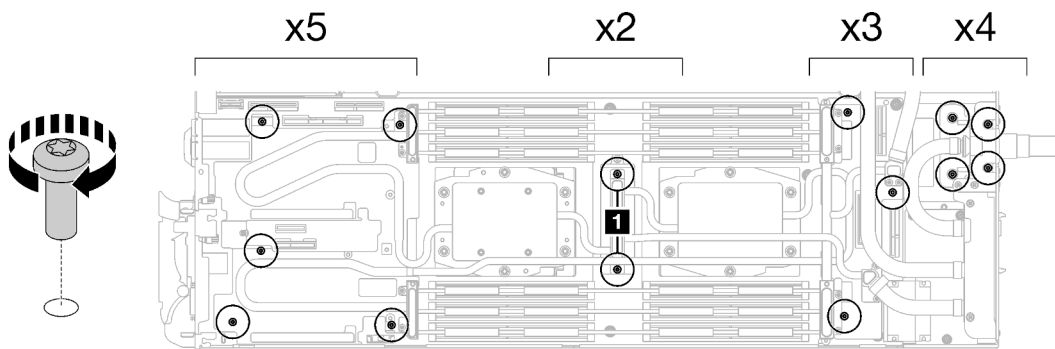
Figura 205. Instalación de los tornillos y tornillos de conexión rápida del bucle de agua
