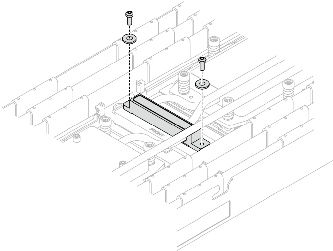
Figura 185. Tornillos de la placa de frío del VR con arandela
