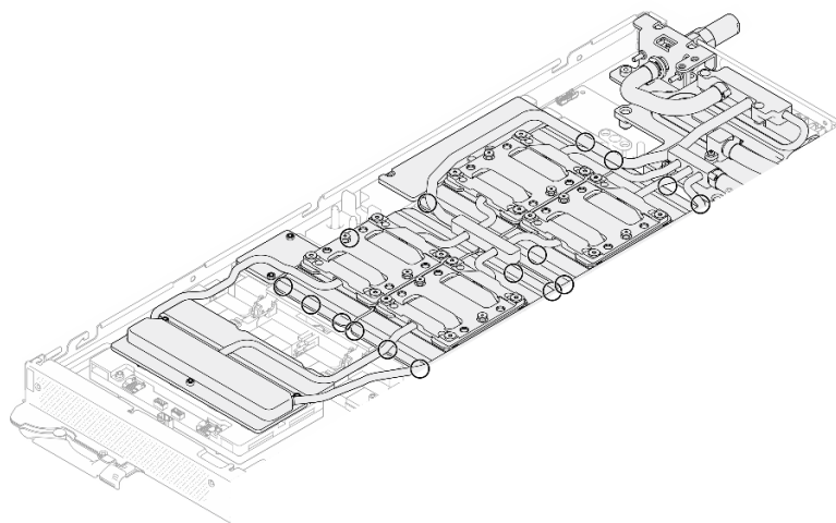
Figura 329. Muecas para soltar las placas de frío de la GPU
