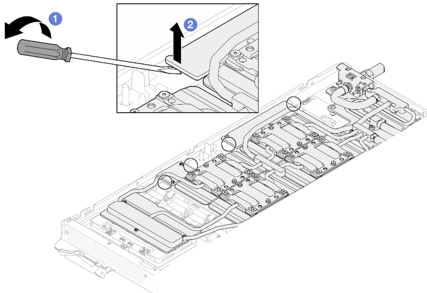
Figura 388. Las placas de conducción MISC delantera y trasera se sueltan ligeramente de la placa de la GPU
