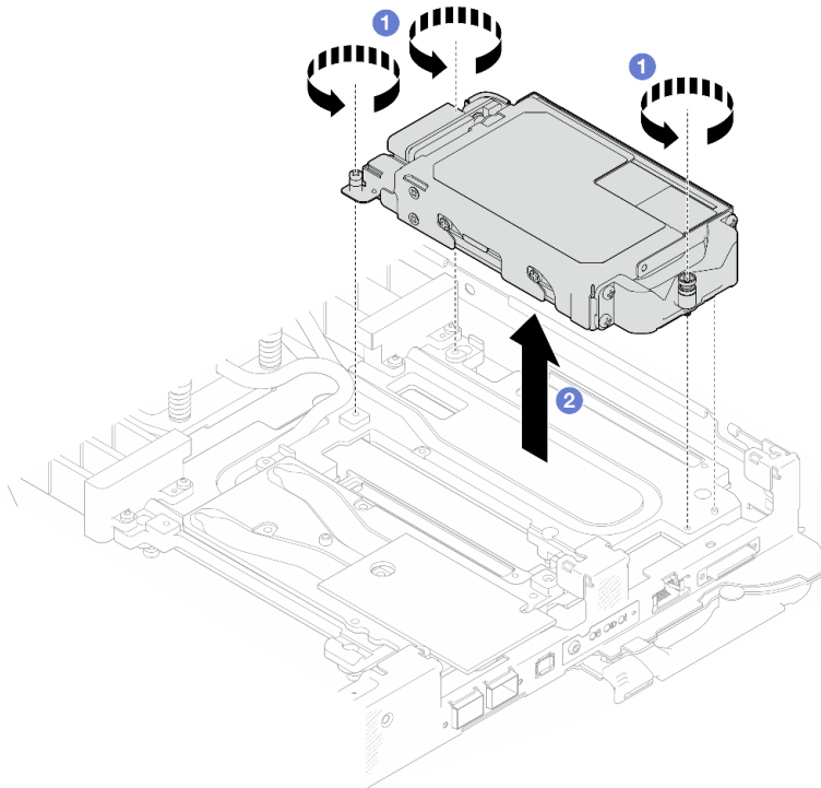
Figura 122. Extracción del conjunto del compartimiento de unidad E3.S
