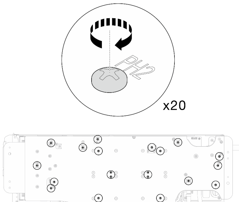
Figura 22. Extracción del tornillo del bucle de agua y del tornillo de conexión rápida (nodo de la GPU)
