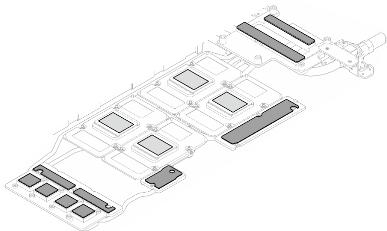
Figura 47. Sustitución de almohadillas de masilla del bucle de agua (nodo de GPU)
