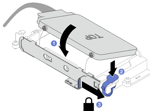
Figura 99. Instalación de la unidad superior (unidad de 7 mm)
