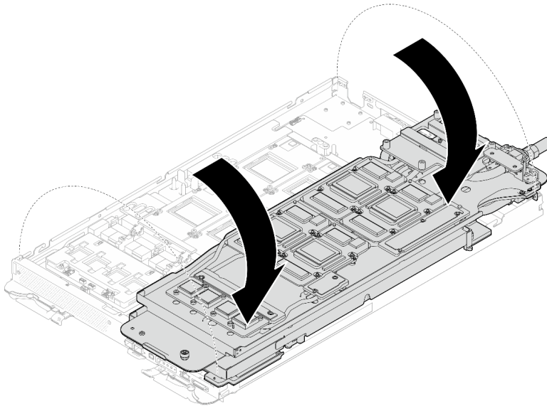
Figura 427. Plegado del bucle de agua del lado del nodo de la GPU en el bucle de agua del lado del nodo de cálculo
