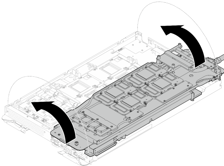
Figura 26. Girar el bucle de agua del nodo de la GPU al nodo de la GPU
