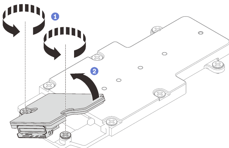
Figura 144. Desmontaje del conjunto de placas posteriores de M.2
