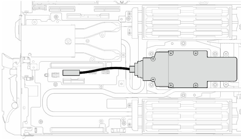
Figura 142. Extracción del cable del conjunto de placas posteriores de M.2
