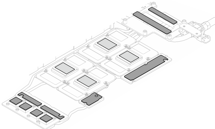
Figura 402. Sustitución de almohadillas de masilla del bucle de agua (nodo de GPU)
