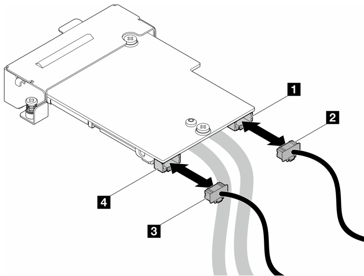
Figura 175. Instalación de los cables de alimentación del módulo OSFP
