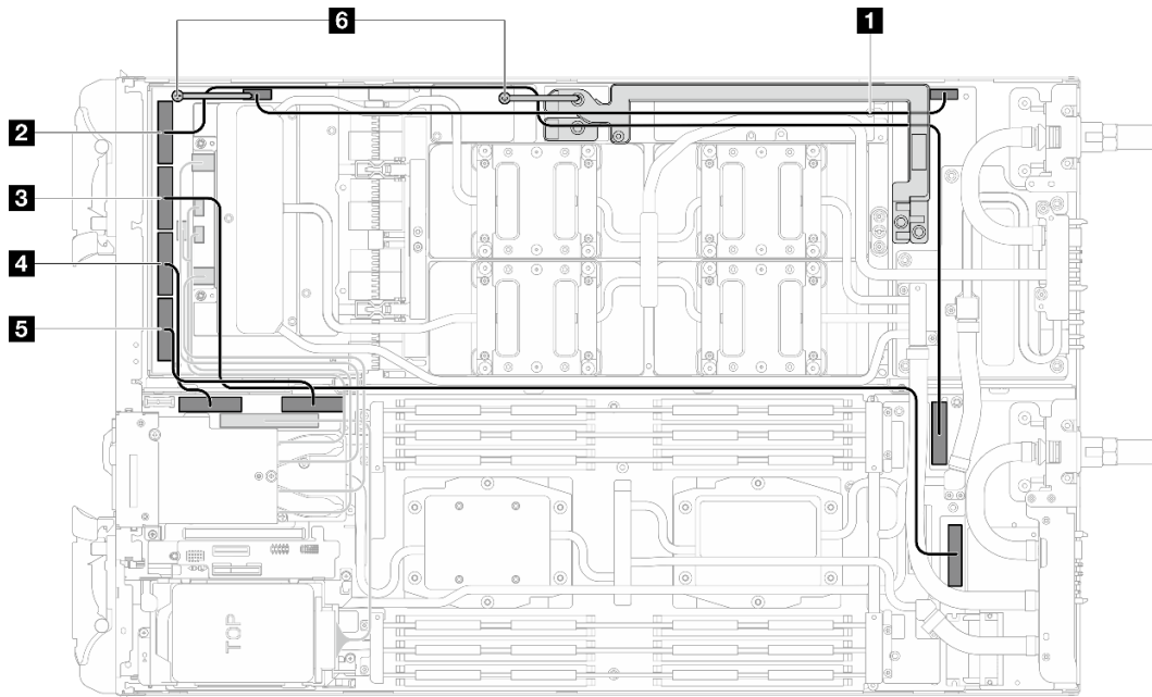
Figura 453. Disposición de los cables para una configuración de dos procesadores
