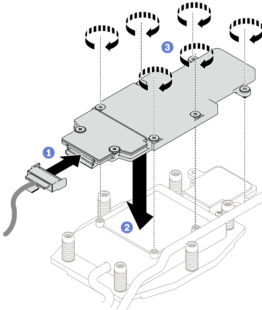
Figura 150. Instalación del conjunto de placas posteriores de M.2
