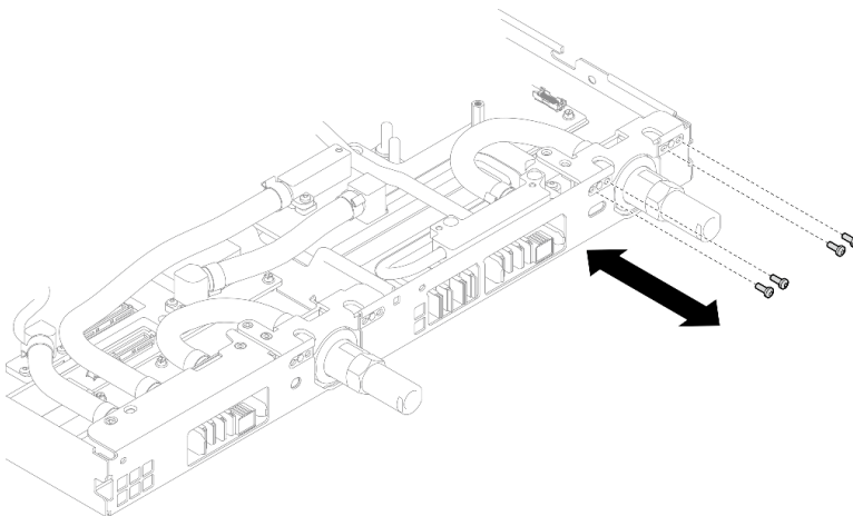
Figura 348. Instalación del tornillo de conexión rápida (nodo de la GPU)
