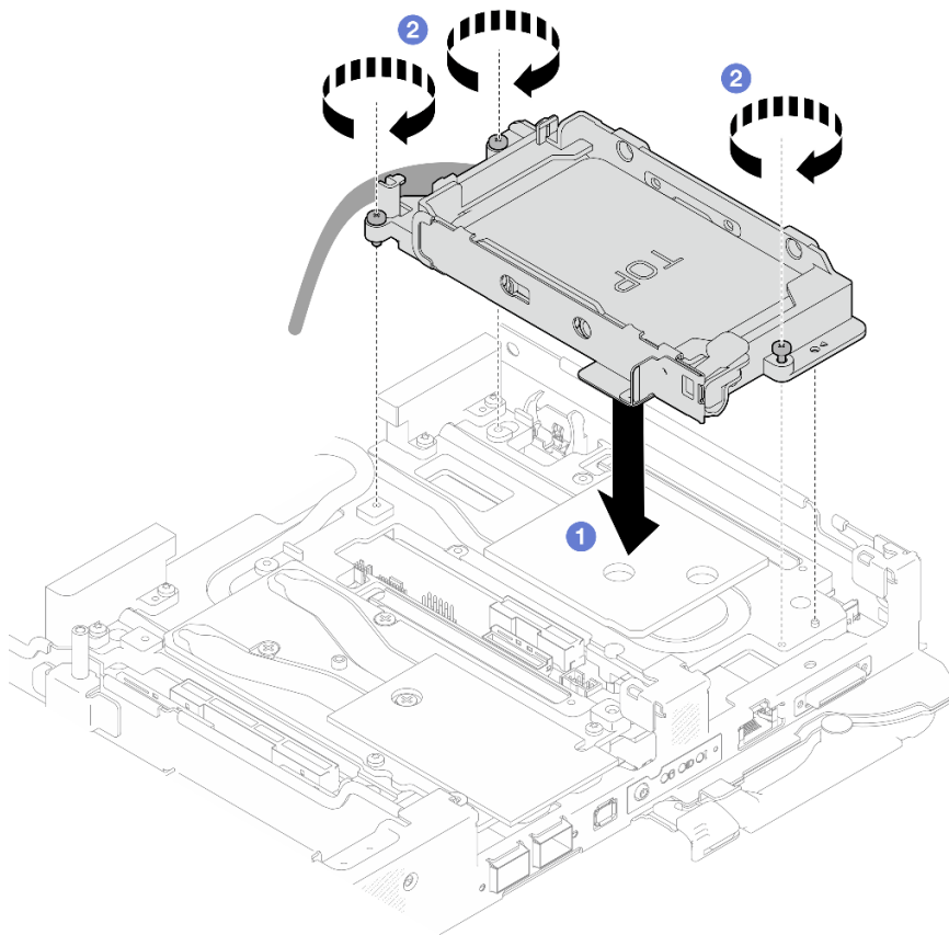
Figura 104. Instalación de un conjunto de compartimiento de la unidad de 7 mm
