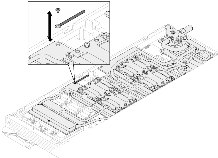
Figura 67. Instalación de la brida de cables
