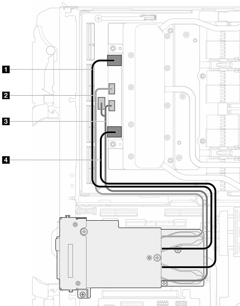
Figura 170. Desconexión de los cables del módulo OSFP de la placa de red
