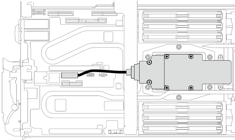
Figura 151. Instalación del cable del conjunto de placas posteriores de M.2
