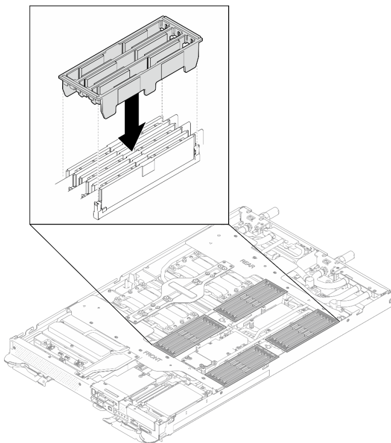
Figura 164. Instalación de la cubierta DIMM
