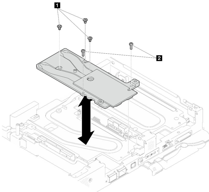
Figura 28. Extracción de la placa de conducción de Módulo OSFP
