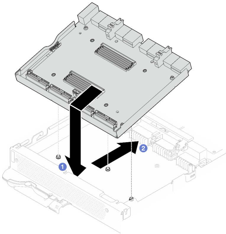
Figura 316. Instalación de la placa del transportador
