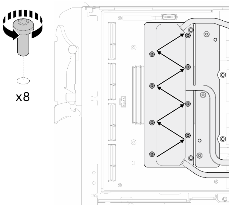
Figura 16. Extracción del tornillo de la tarjeta de red
