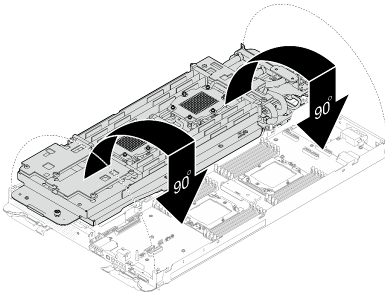
Figura 260. Instalación del bucle de agua
