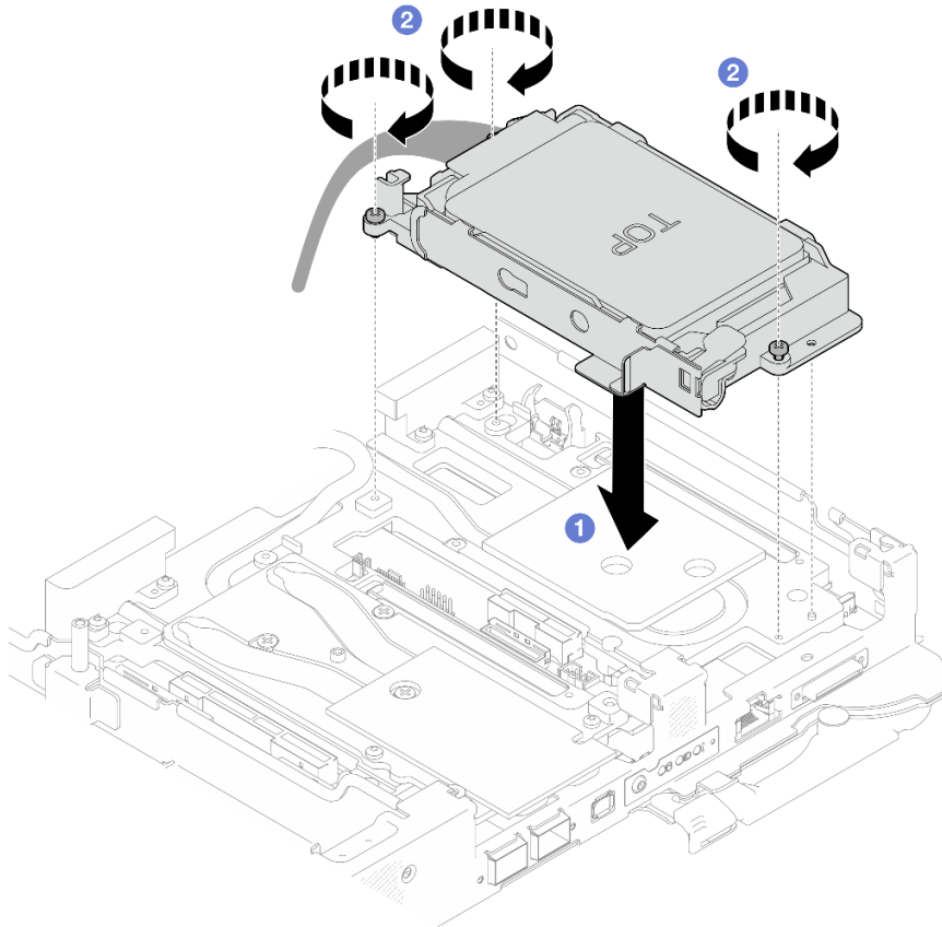
Figura 105. Instalación de dos conjuntos de compartimiento de la unidad de 7 mm
