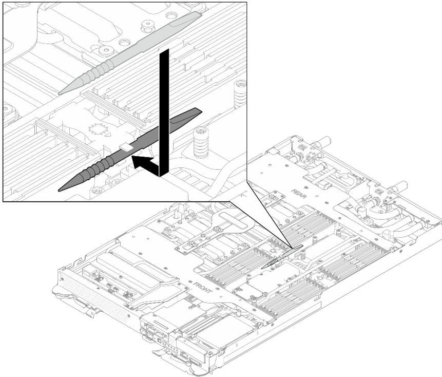
Figura 165. Herramienta del módulo de memoria
