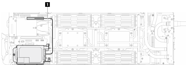
Figura 167. Desconexión del cable de la unidad E3.s
