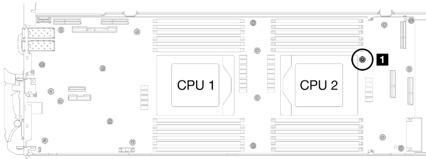
Figura 300. Ubicación del orificio de tornillo del cable protector 4
