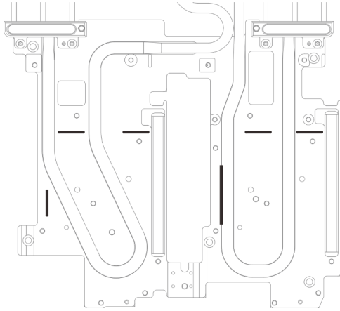
Figura 102. Marcas en el bucle de agua para la alineación de la almohadilla de espacio
