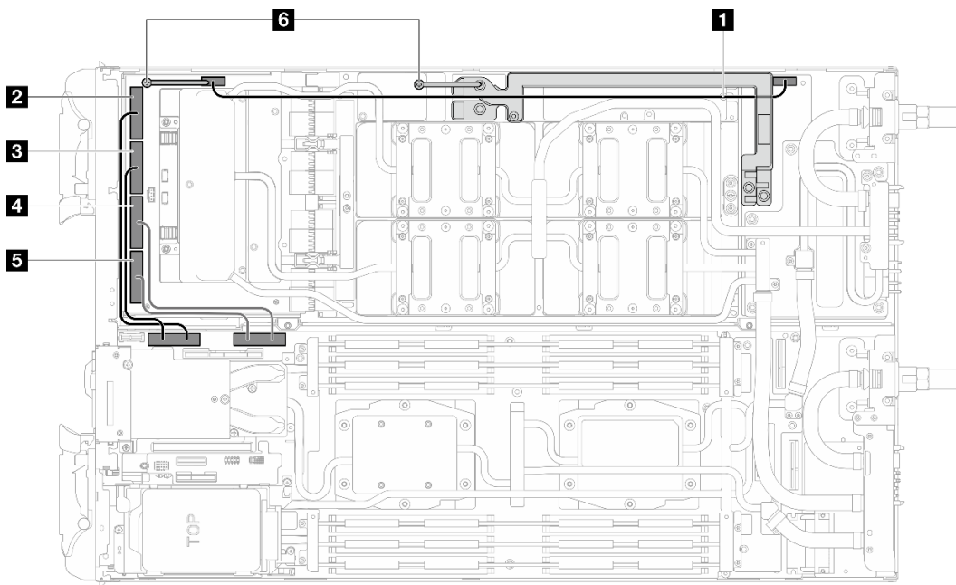
Figura 452. Disposición de los cables para una configuración de un procesador
