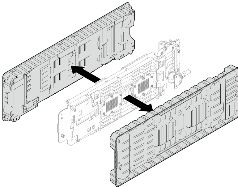
Figura 255. Extracción de las cubiertas de plástico para grasa
