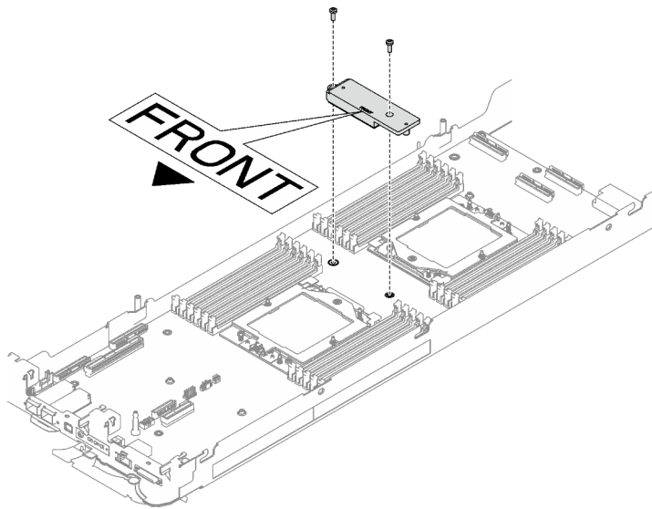
Figura 78. Extracción de la placa de conducción del VR
