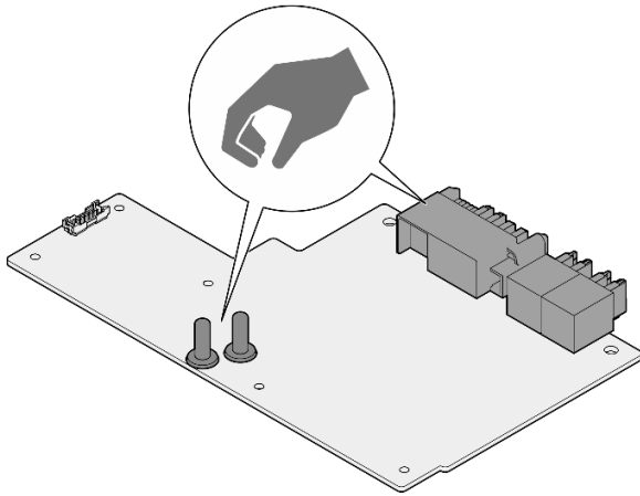
Figura 380. Puntos de contacto de la placa de distribución de alimentación de la GPU de SD665-N V3
