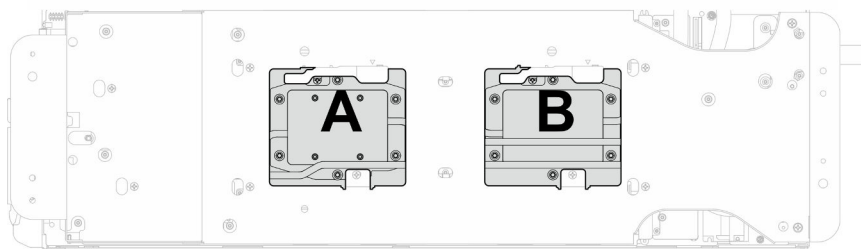
Figura 234. Instalación de la placa de frío del procesador
