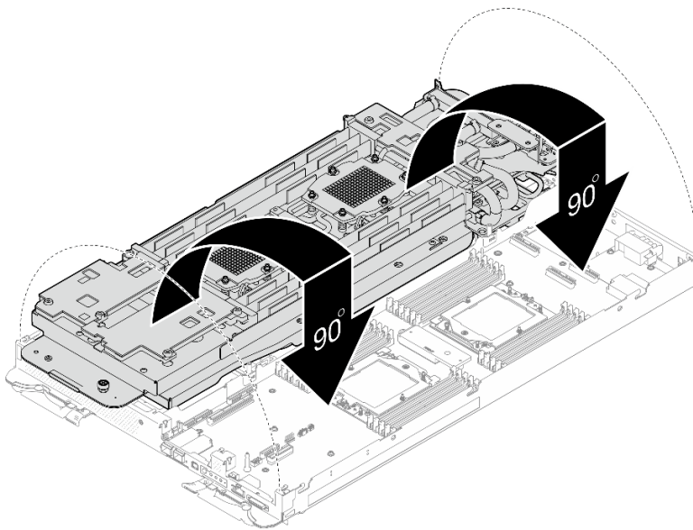
Figura 200. Instalación del bucle de agua
