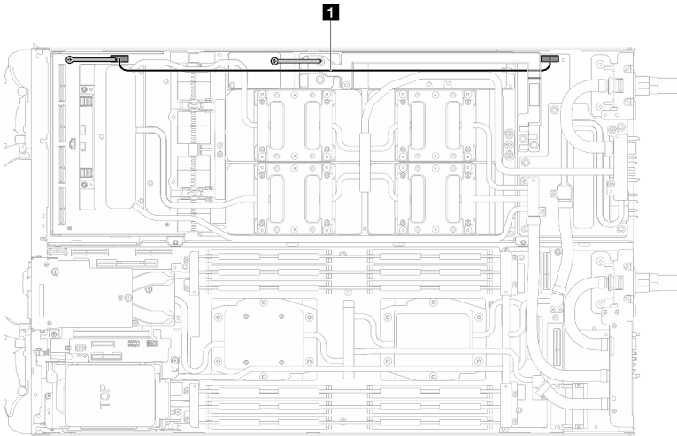
Figura 319. Conexión del cable de alimentación de la placa del transportador
