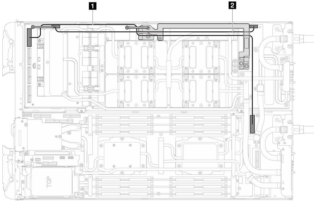
Figura 310. Disposición del cable de alimentación y del cable MCIO 1 de la placa del transportador
