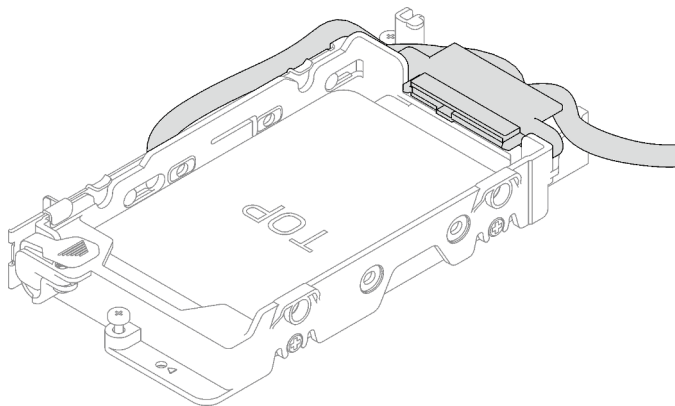
Figura 96. Fijación del conector del cable no conectado
