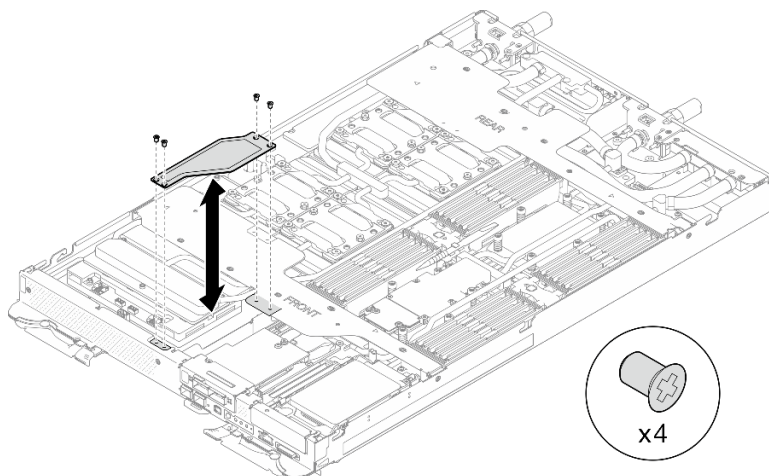
Figura 10. Instalación de la cubierta de cables frontal
