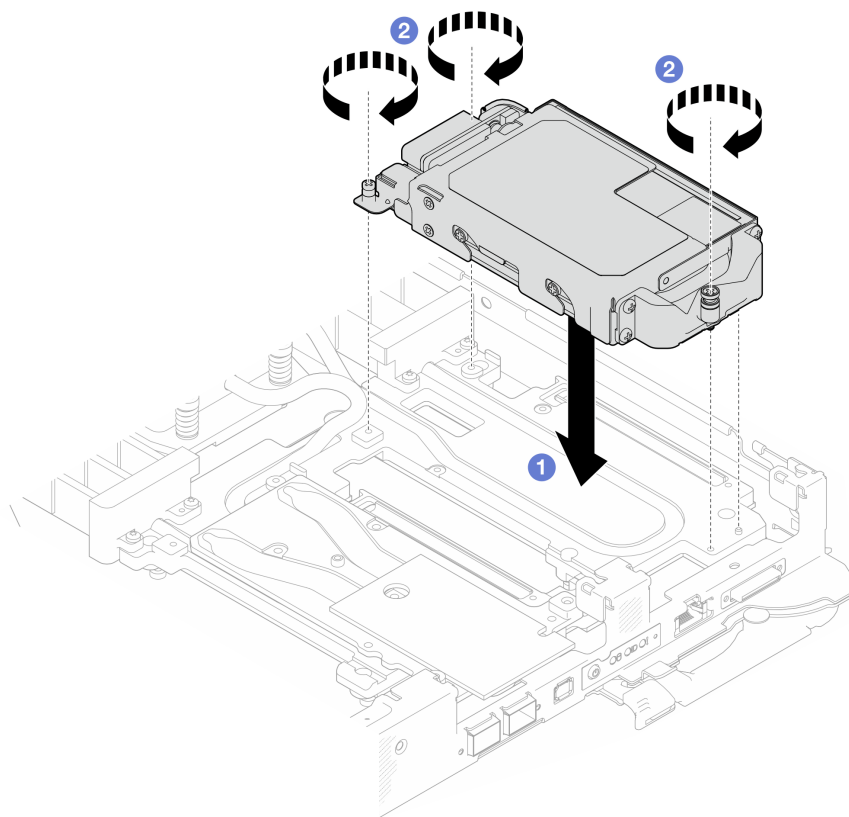
Figura 140. Instalación de un conjunto de compartimiento de una unidad E3.S
