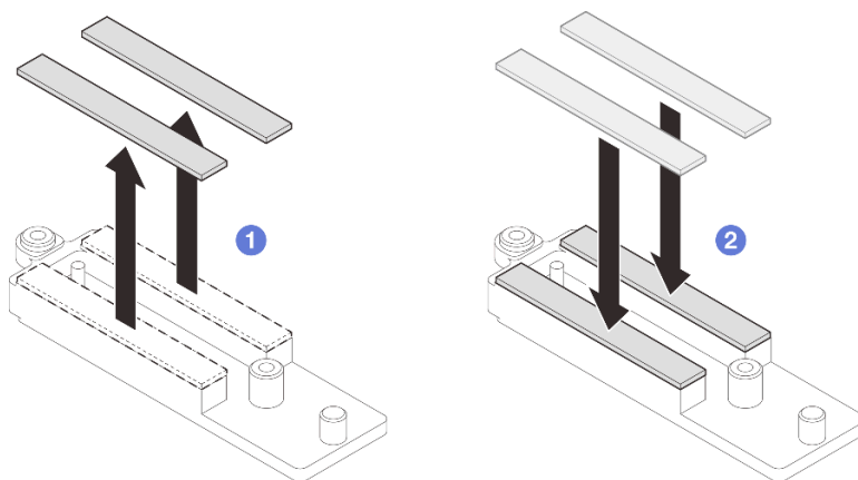
Figura 295. Sustitución de las almohadillas de masilla de la placa de conducción de VR
