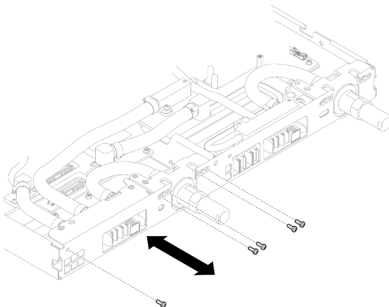
Figura 243. Extracción del tornillo de la conexión rápida (nodo de cálculo)
