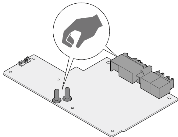
Figura 398. Puntos de contacto de la placa de distribución de alimentación de la GPU de SD665-N V3
