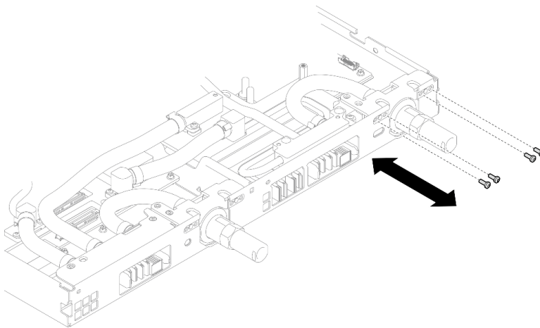
Figura 442. Instalación del tornillo de conexión rápida (nodo de la GPU)
