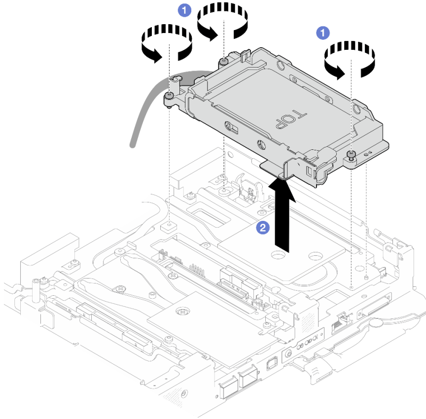
Figura 88. Quitar un conjunto de compartimiento de la unidad de 7 mm
