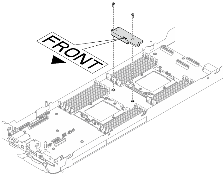
Figura 271. Extracción de la placa de conducción del VR
