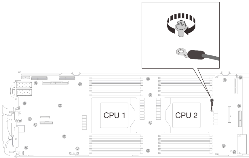
Figura 301. Instalación del cable protector 4
