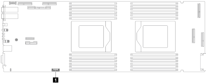
Figura 81. Ubicación de batería CMOS
