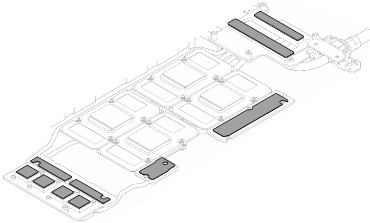
Figura 25. Limpieza de las almohadillas de masilla del bucle de agua
