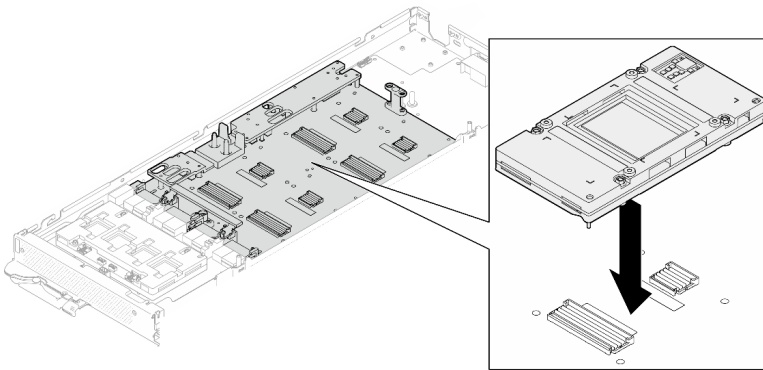
Figura 338. Instalación de la GPU
