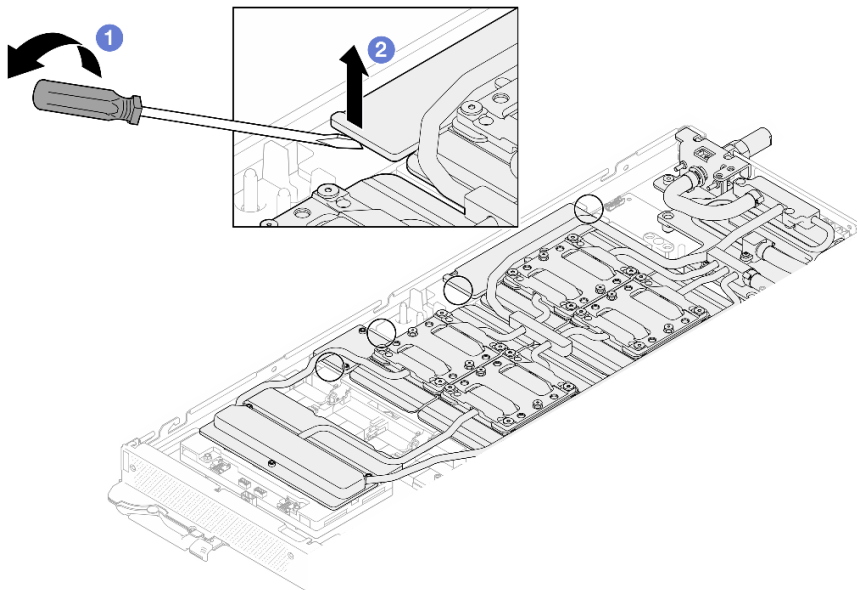
Figura 422. Las placas de conducción MISC delantera y trasera se sueltan ligeramente de la placa de la GPU
