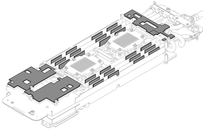
Figura 227. Almohadillas de espacio del bucle de agua (parte inferior)
