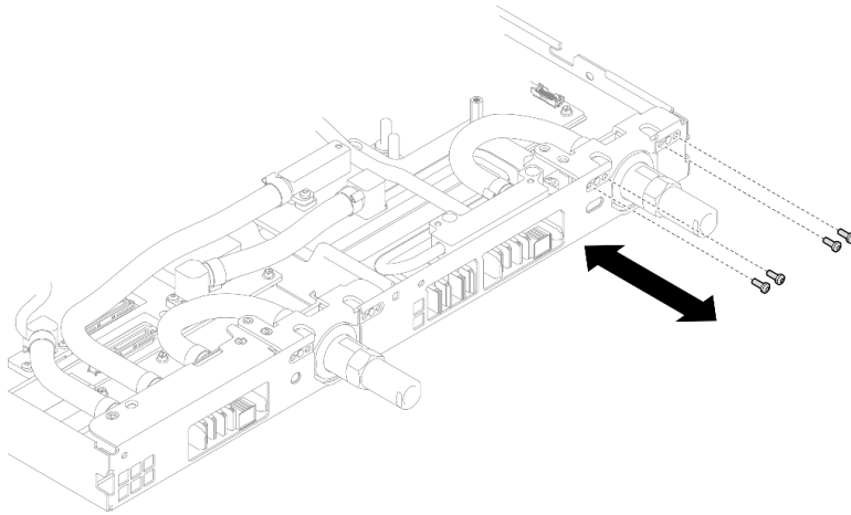
Figura 64. Instalación del tornillo de conexión rápida (nodo de la GPU)
