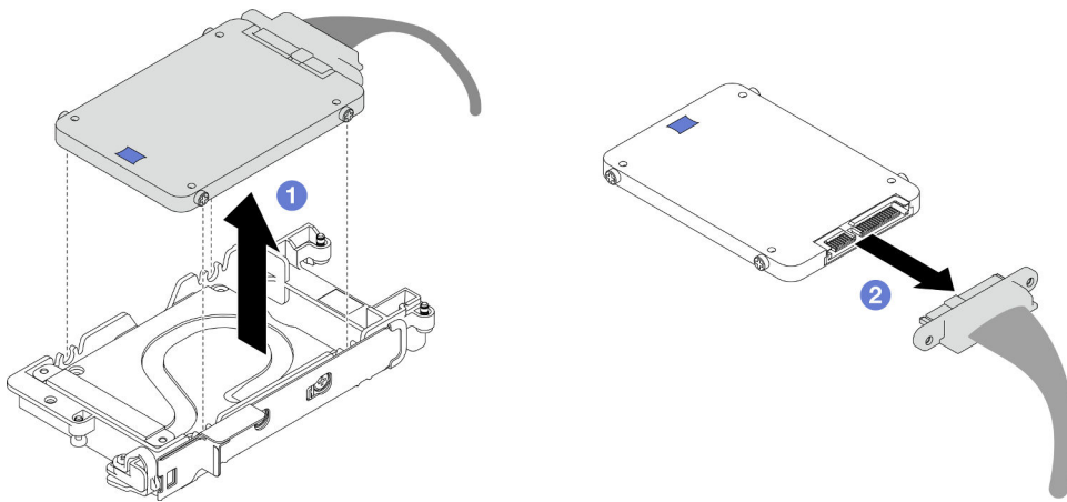
Figura 111. Extracción de la unidad inferior
