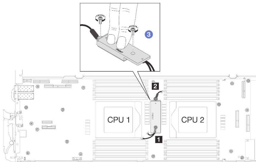
Figura 282. Instalación del cable protector 1/2 y 3
