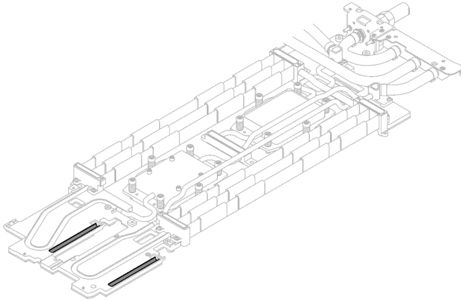
Figura 197. Almohadillas de espacio del bucle de agua (parte superior)
