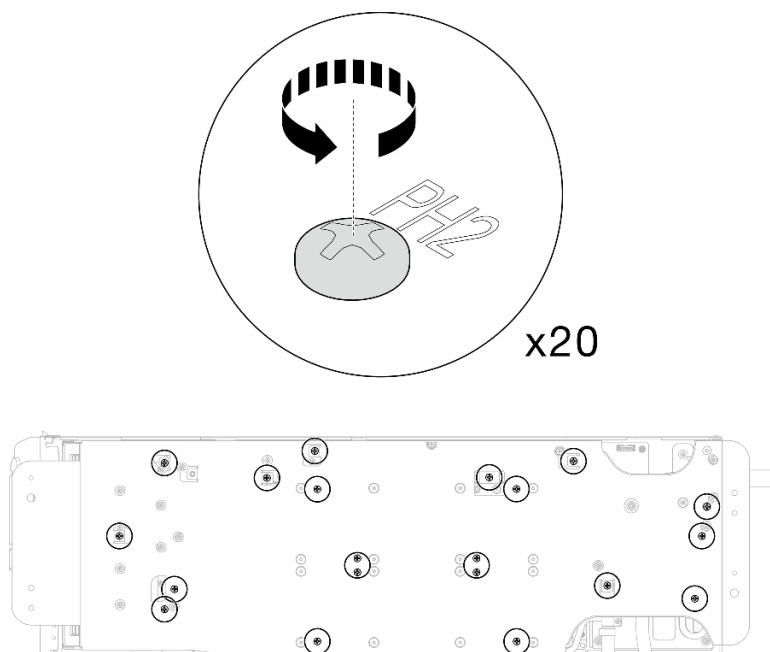
Figura 60. Instalación de los tornillos y tornillos de conexión rápida del bucle de agua (nodo de la GPU)
