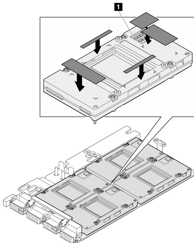
Figura 436. Sustitución de las almohadillas de masilla de la GPU
