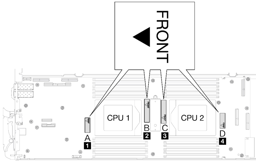
Figura 289. Marcación frontal en el compartimiento que apunta a la parte frontal
