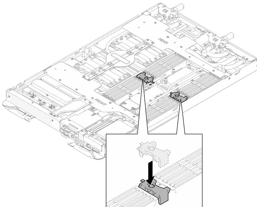
Figura 85. Instalación de la guía del DIMM
