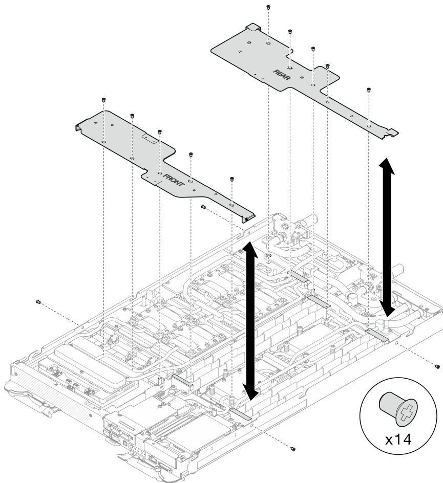
Figura 9. Instalación de las llaves cruzadas frontales y traseras
