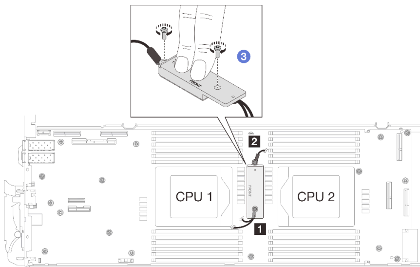
Figura 299. Instalación del cable protector 1/2 y 3
