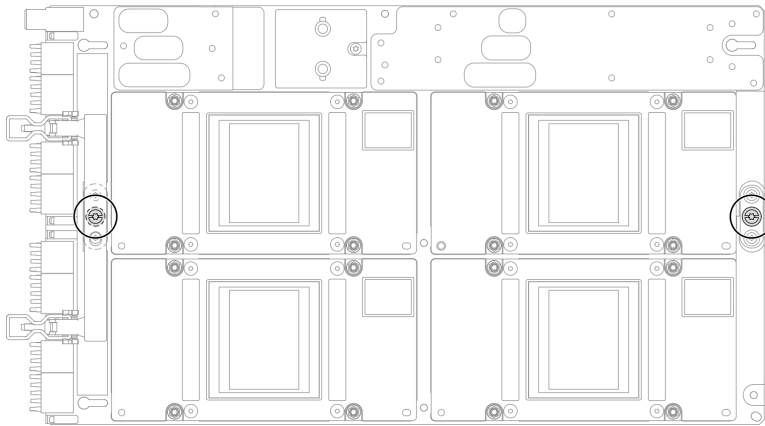
Figura 376. Instalación de los tornillos T15 en el conjunto de la placa de la GPU
