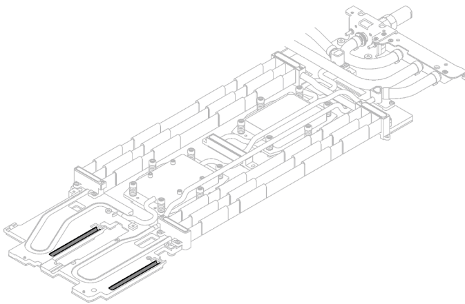
Figura 257. Almohadillas de espacio del bucle de agua (parte superior)
