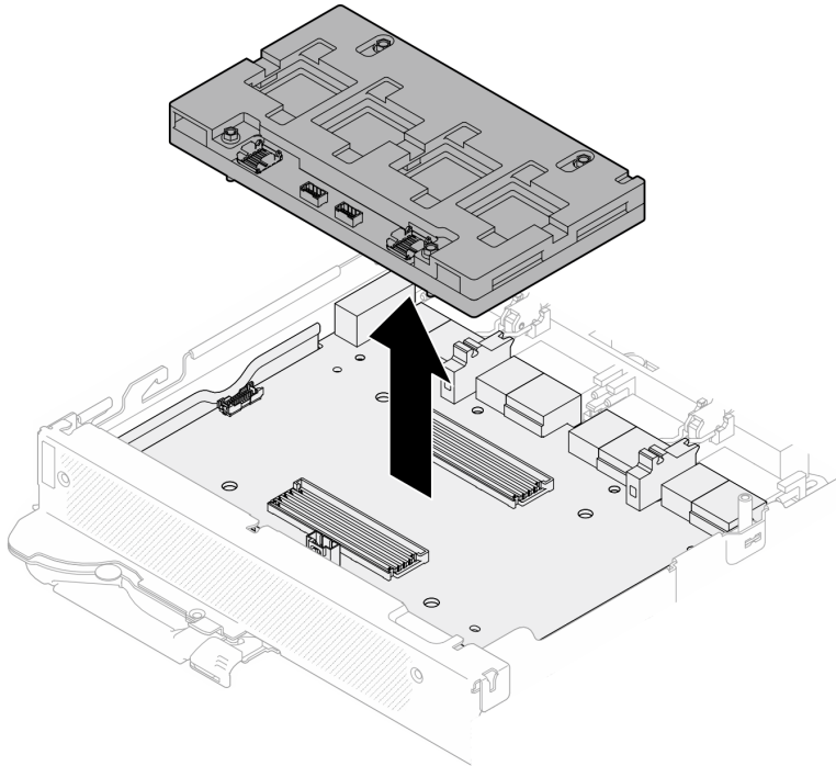
Figura 431. Extracción la placa de red
