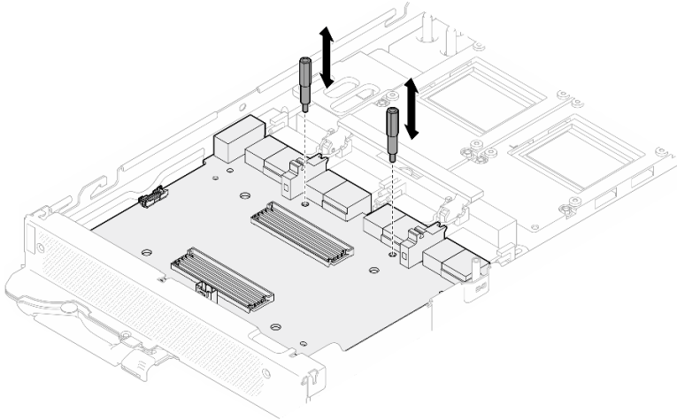
Figura 318. Instalación de los aisladores de la placa del transportador
