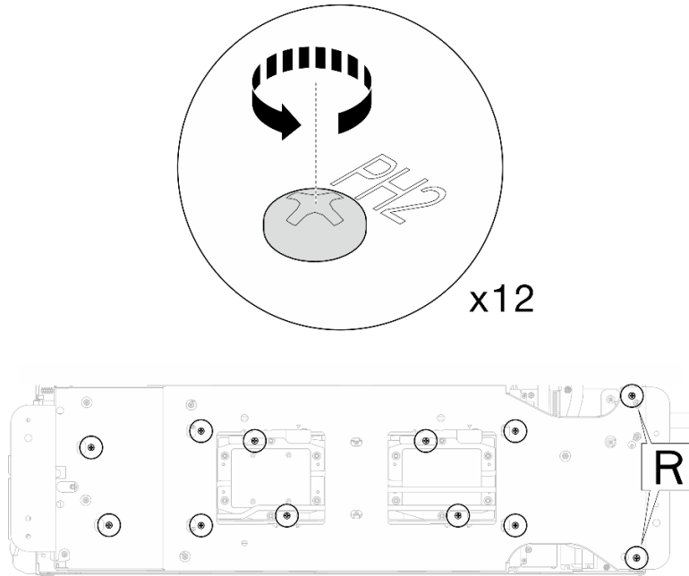
Figura 51. Soltar los tornillos del transportador del bucle de agua
