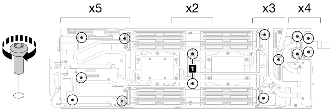
Figura 236. Instalación de los tornillos y tornillos de conexión rápida del bucle de agua
