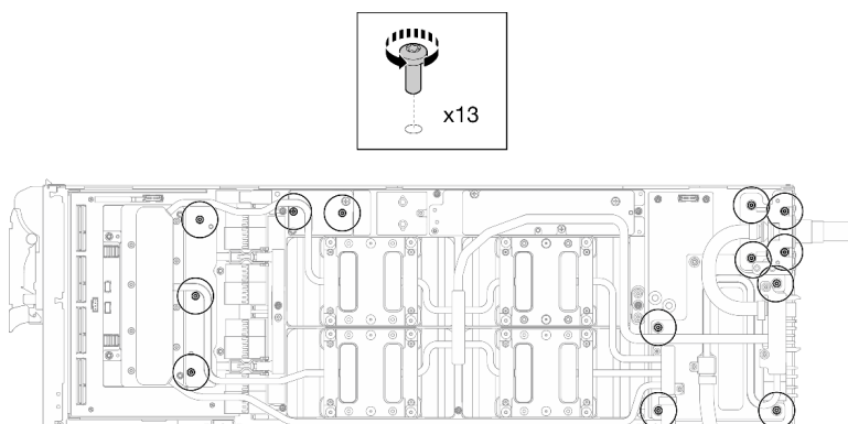
Figura 418. Extracción de los tornillos Torx T10 del bucle de agua (nodo de la GPU)
