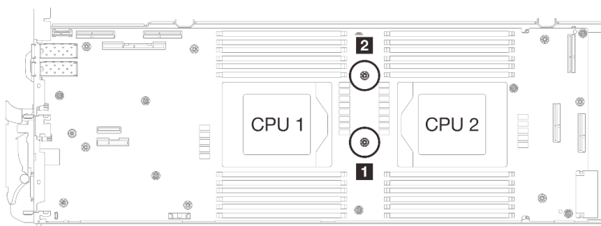
Figura 71. Ubicación de los orificios de tornillo del cable protector 1/2 y 3
