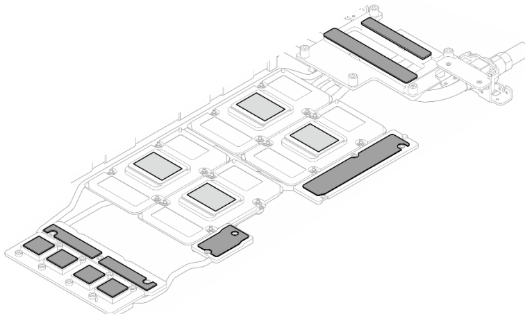
Figura 435. Sustitución de almohadillas de masilla del bucle de agua (nodo de GPU)
