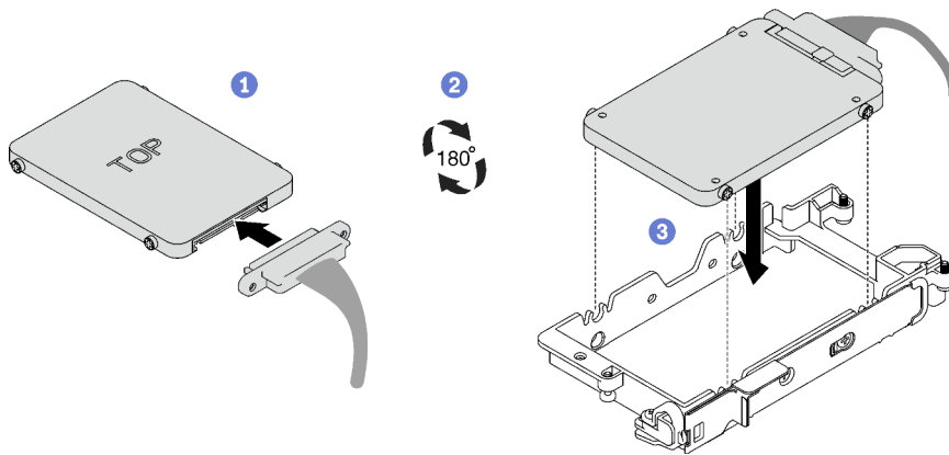
Figura 95. Instalación de la unidad de 7 mm
