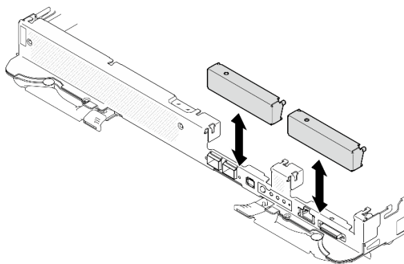
Figura 123. Extracción del relleno vacío del marco biselado
