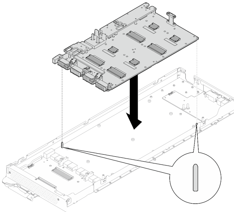
Figura 361. Instalación de la placa de la GPU
