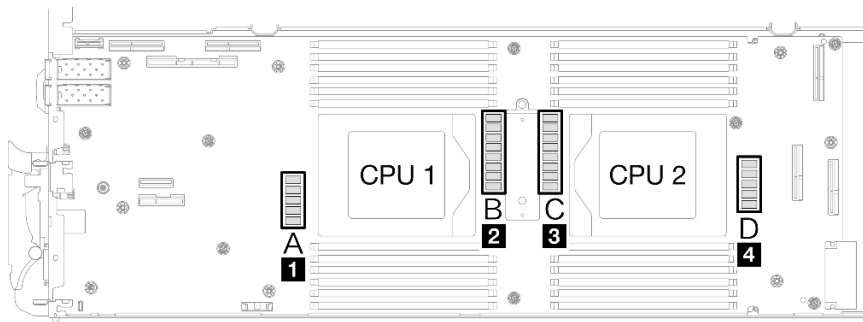
Figura 288. Ubicaciones de los inductores en la placa del sistema
