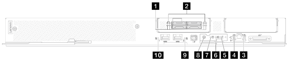
Figura 457. LED frontales de la bandeja SD665-N V3
