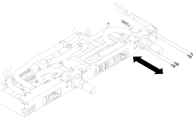
Figura 409. Instalación del tornillo de conexión rápida (nodo de la GPU)
