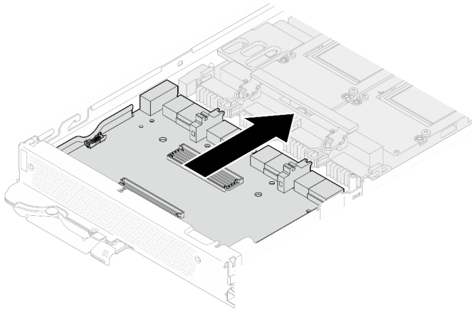
Figura 364. Conexión de la placa del transportador a la placa de la GPU.
