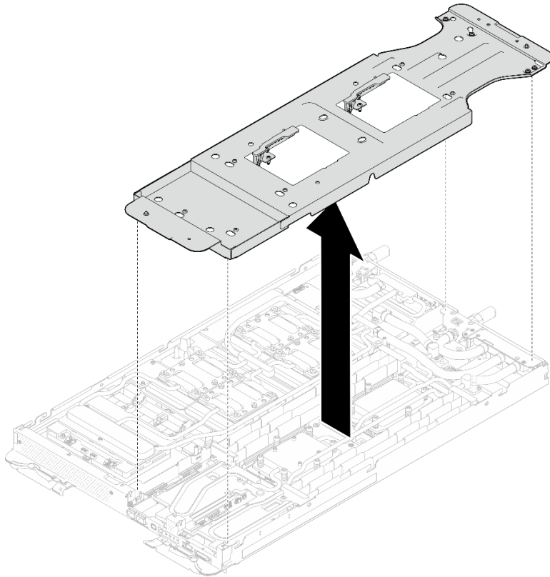
Figura 202. Extracción del transportador del bucle de agua (nodo de cálculo)
