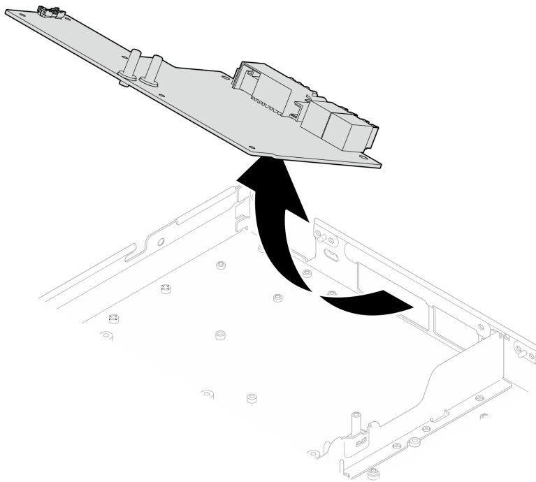
Figura 397. Extracción de la placa de distribución de alimentación de la GPU
