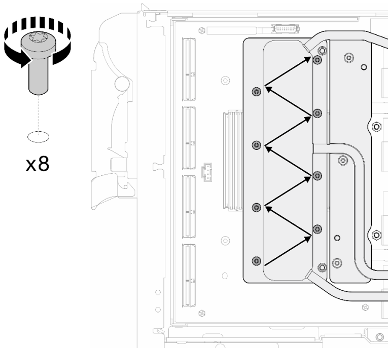
Figura 326. Extracción del tornillo de la tarjeta de red
