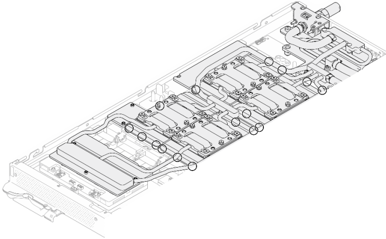
Figura 423. Muecas para soltar las placas de frío de la GPU
