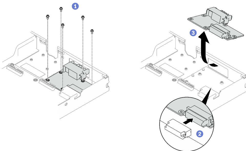
Figura 193. Extracción de la placa de distribución de alimentación
