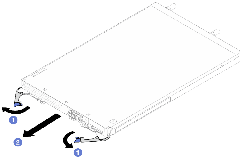
Figura 3. Extracción de la bandeja
