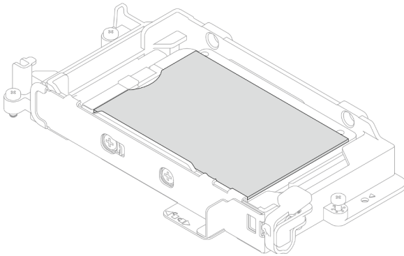
Figura 112. Instalación de la almohadilla de espacio de la placa de conducción
