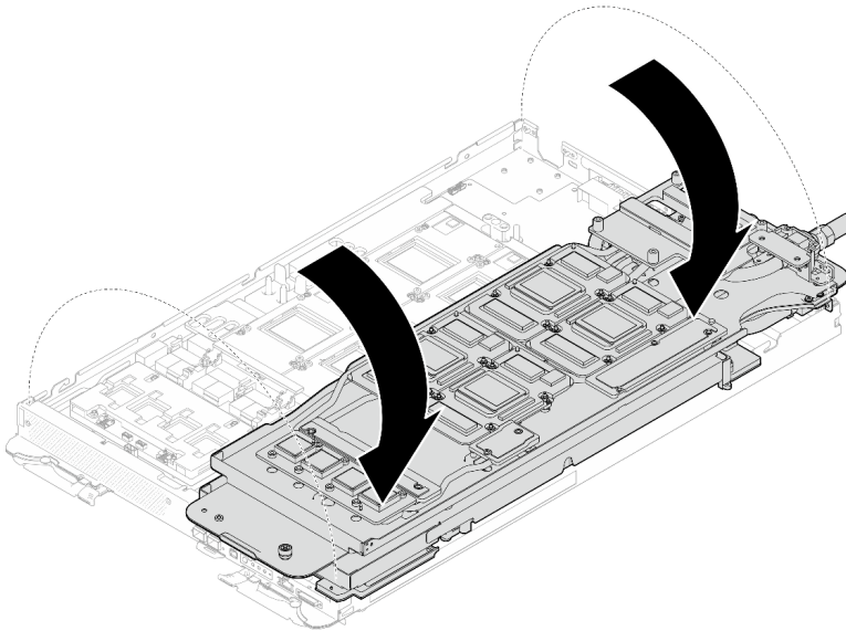
Figura 23. Plegado del bucle de agua del lado del nodo de la GPU en el bucle de agua del lado del nodo de cálculo
