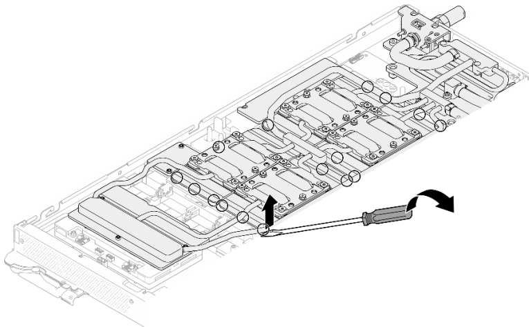
Figura 20. Liberación de la placa de frío de la GPU desde la GPU
