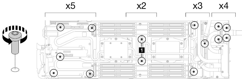
Figura 186. Extracción del tornillo del bucle de agua
