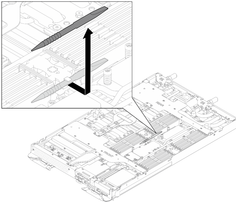
Figura 160. Extracción de la herramienta del módulo de memoria
