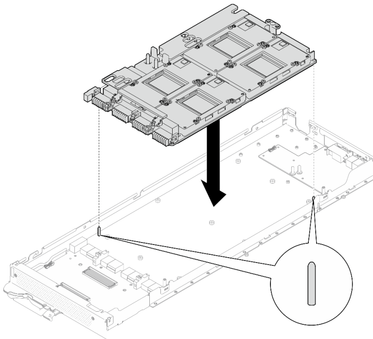
Figura 374. Instalación del conjunto de la placa de la GPU en el nodo
