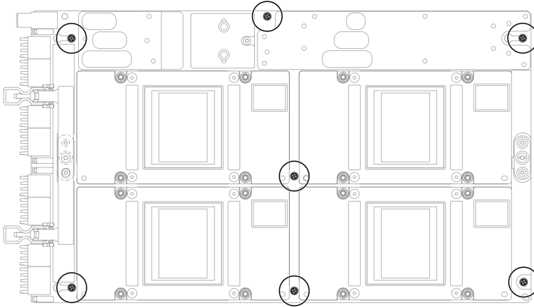
Figura 370. Extracción de los tornillos M3 del conjunto de la placa de la GPU
