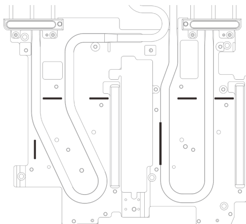
Figura 117. Marcas en el bucle de agua para la alineación de la almohadilla de espacio
