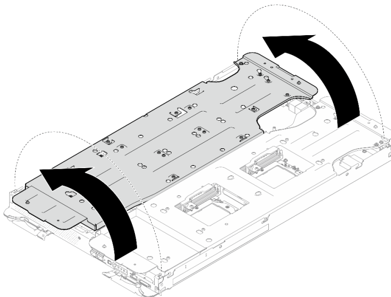
Figura 50. Desdoblar el bucle de agua
