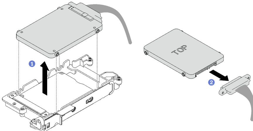
Figura 93. Extracción de la unidad inferior
