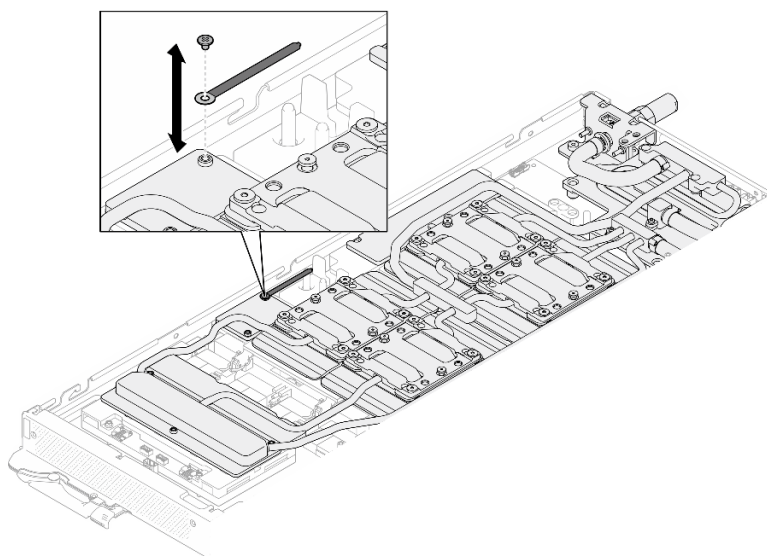
Figura 416. Extracción de la brida de cables
