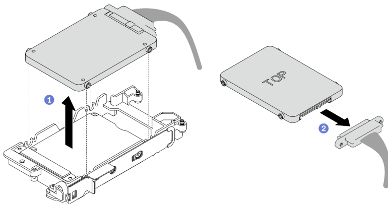
Figura 91. Extracción de una unidad de 7 mm
