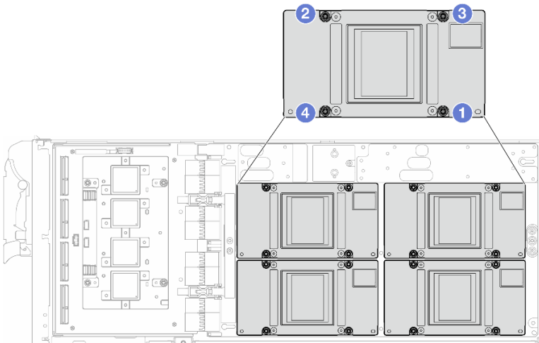
Figura 339. Secuencia de apriete de los tornillos de la GPU
