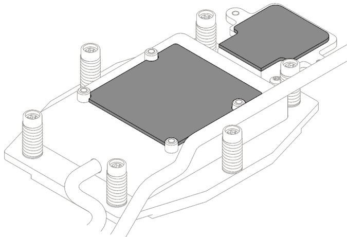
Figura 149. Almohadillas de masilla en la placa de frío del procesador y placa de frío de M.2
