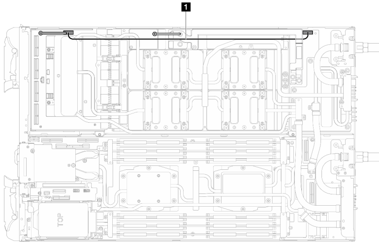
Figura 381. Extracción del cable de alimentación de la placa del transportador
