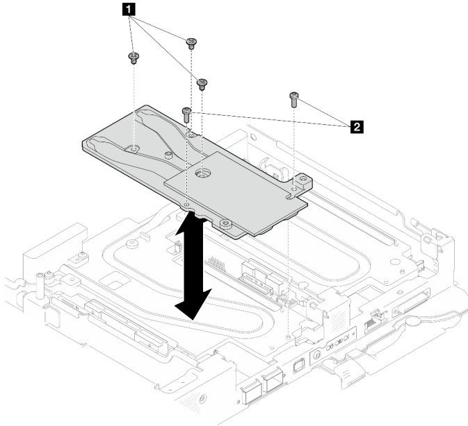
Figura 58. Instalación de la placa de conducción del Módulo OSFP
