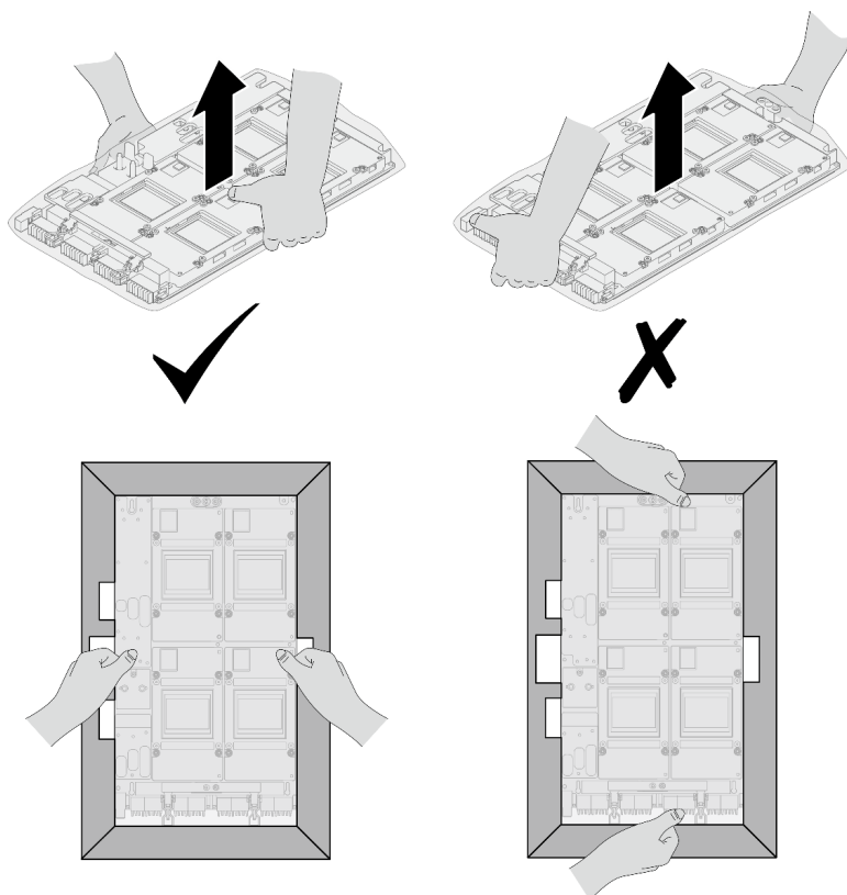
Figura 372. Extracción del conjunto de la placa de la GPU de la caja del paquete
