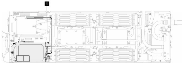
Figura 181. Conexión del cable de la unidad E3.s
