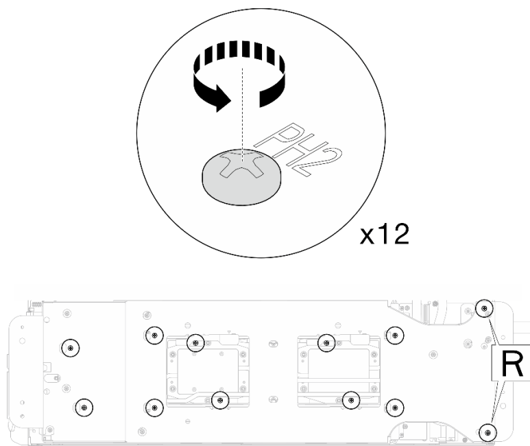
Figura 261. Soltar los tornillos del transportador del bucle de agua
