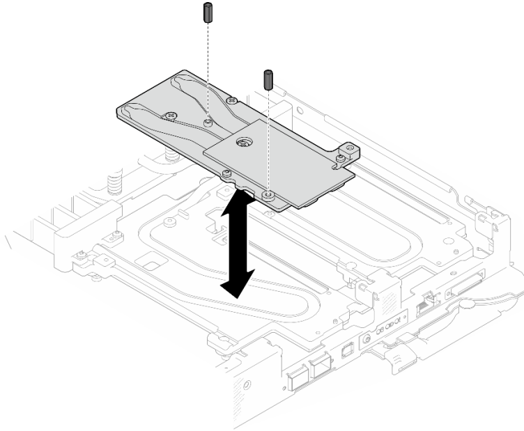
Figura 211. Extracción de los tornillos hexagonales de la placa de conducción de Módulo OSFP
