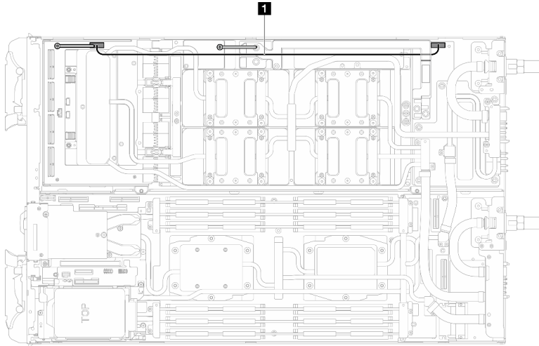
Figura 68. Conexión del cable de alimentación de la placa del transportador
