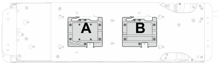
Figura 53. Instalación de la placa de frío del procesador
