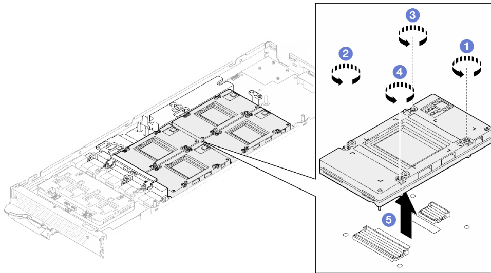
Figura 336. Extracción de la GPU
