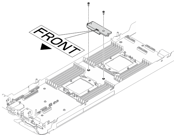
Figura 69. Extracción de la placa de conducción del VR
