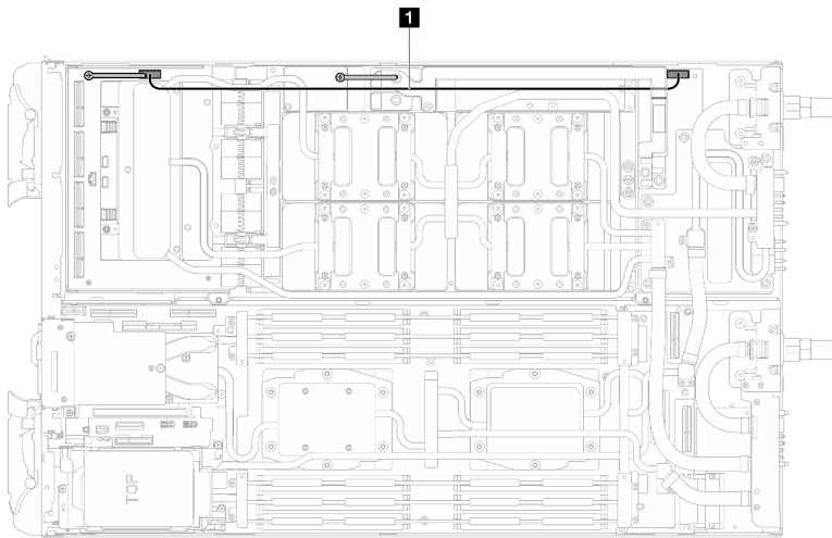
Figura 352. Conexión del cable de alimentación de la placa del transportador
