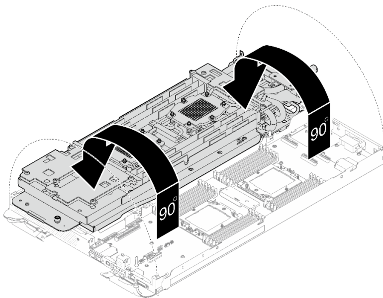
Figura 221. Doblar el bucle de agua
