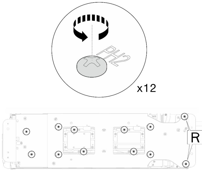
Figura 201. Soltar los tornillos del transportador del bucle de agua
