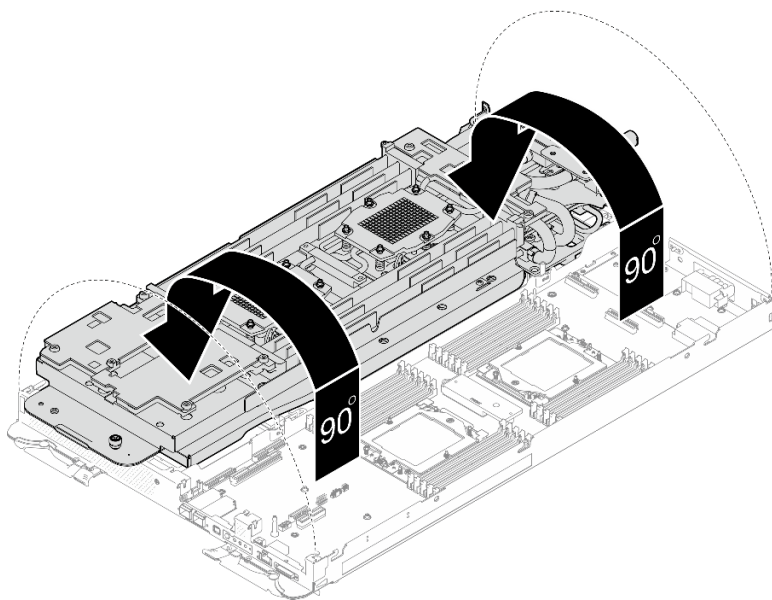
Figura 192. Doblar el bucle de agua
