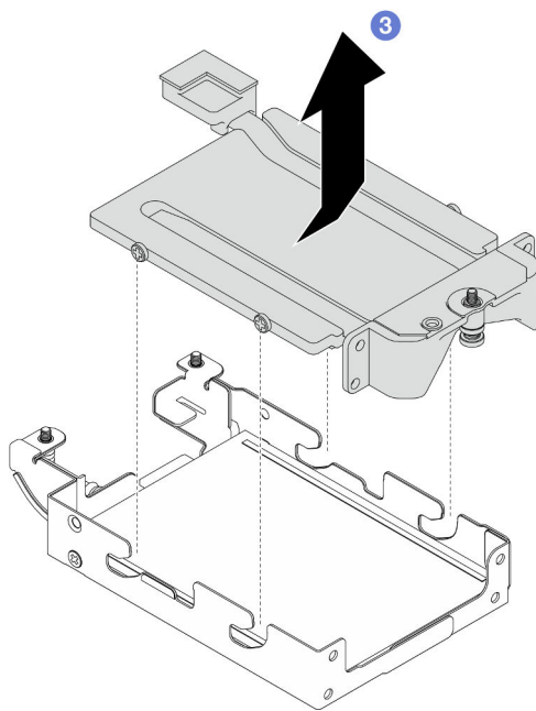
Figura 128. Extracción de la placa de conducción
