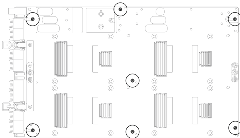
Figura 362. Instalación de los tornillos M3 en la placa de la GPU
