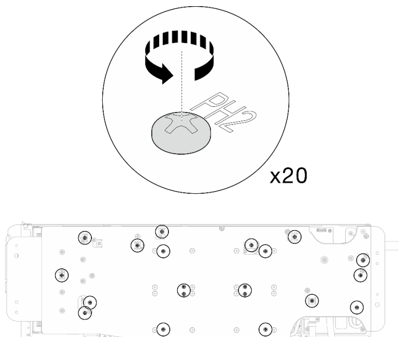
Figura 344. Instalación de los tornillos y tornillos de conexión rápida del bucle de agua (nodo de la GPU)
