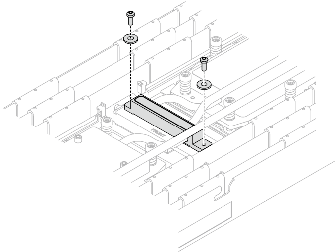
Figura 214. Tornillos de la placa de frío del VR con arandela
