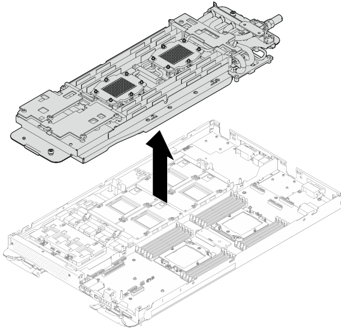
Figura 39. Extracción del bucle de agua
