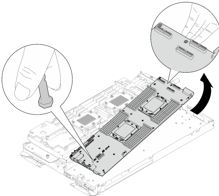
Figura 273. Extracción de la placa del sistema
