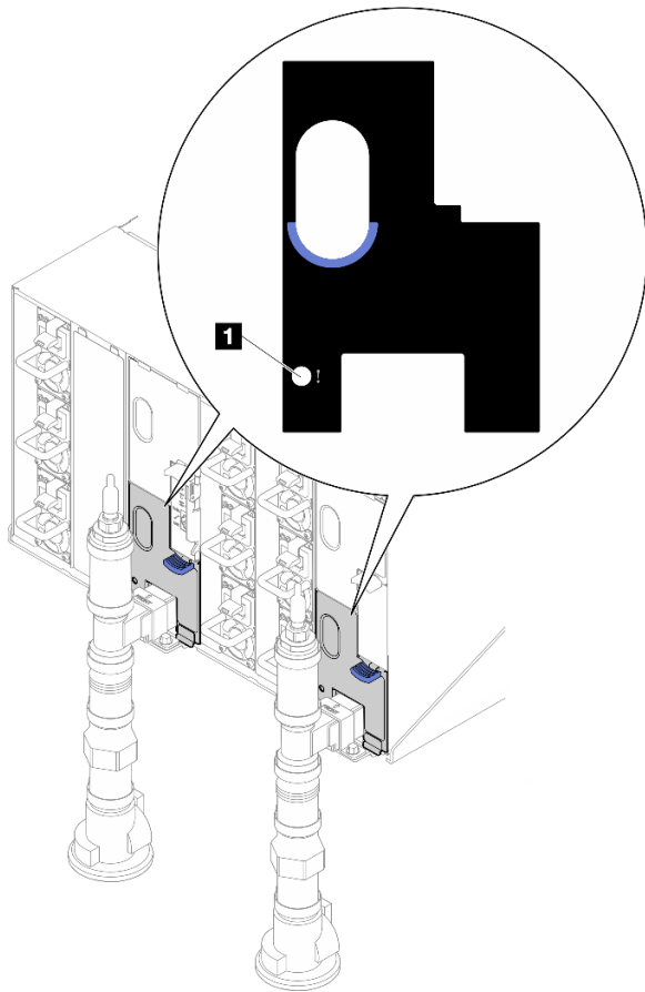
Figura 461. LED de sensor de goteo
