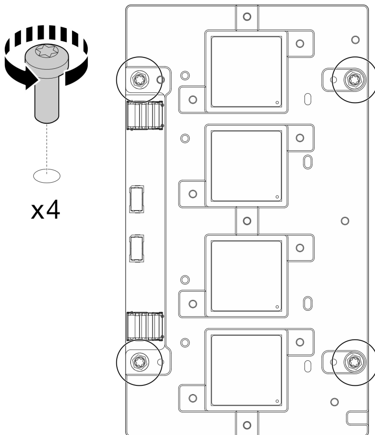
Figura 430. Extracción de los tornillos de la placa de red
