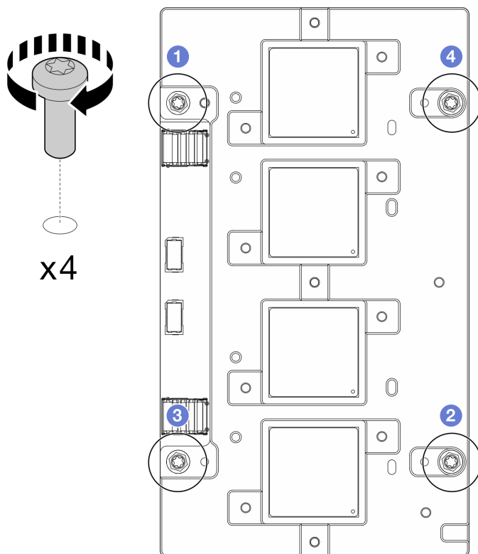
Figura 433. Instalación de los tornillos de la placa de red
