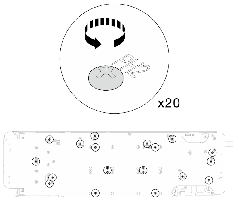
Figura 405. Instalación de los tornillos y tornillos de conexión rápida del bucle de agua (nodo de la GPU)
