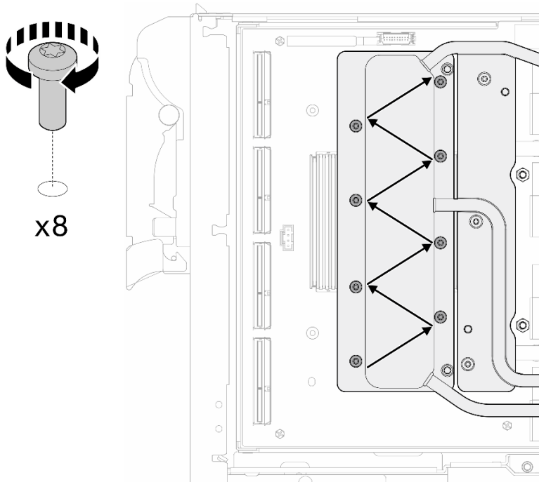
Figura 441. Instalación del tornillo de la tarjeta de red
