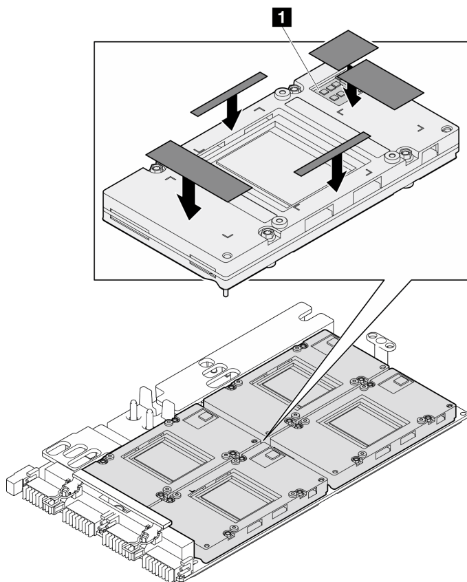
Figura 48. Sustitución de las almohadillas de masilla de la GPU
