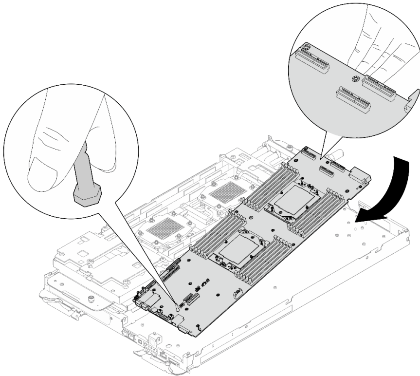
Figura 276. Instalación de la placa del sistema
