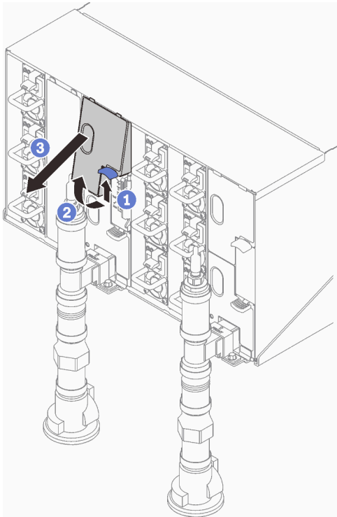
Figura 466. Extracción de la protección EMC superior
