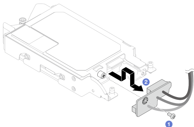
Figura 126. Extracción de la placa posterior con cable de la unidad E3.s
