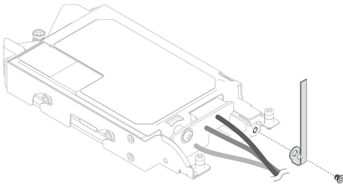
Figura 136. Instalación de la brida de cables
