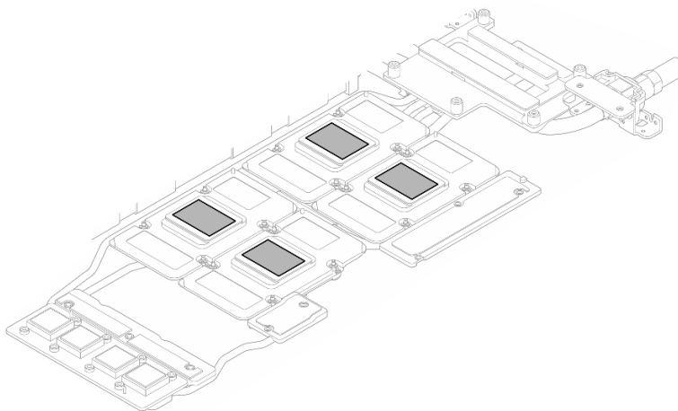
Figura 394. Limpieza del PCM de todas las GPU
