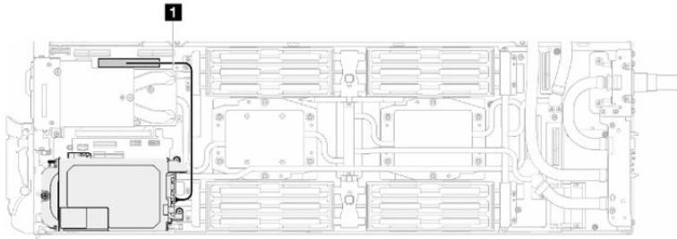
Figura 121. Desconexión del cable de la unidad E3.s
