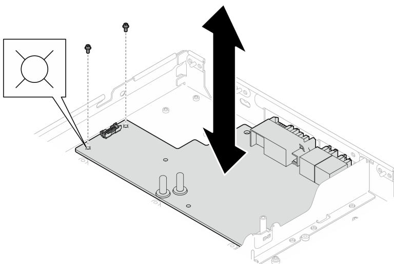
Figura 400. Instalación de los tornillos de la placa de distribución de alimentación de la GPU
