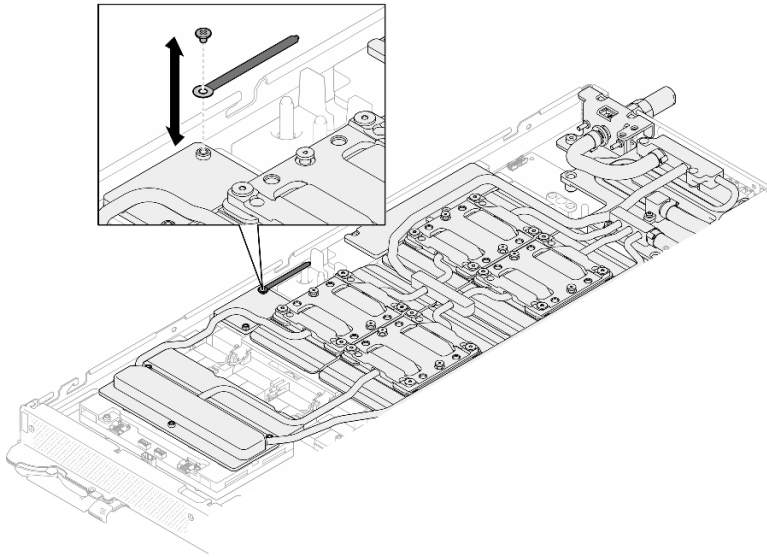
Figura 445. Instalación de la brida de cables
