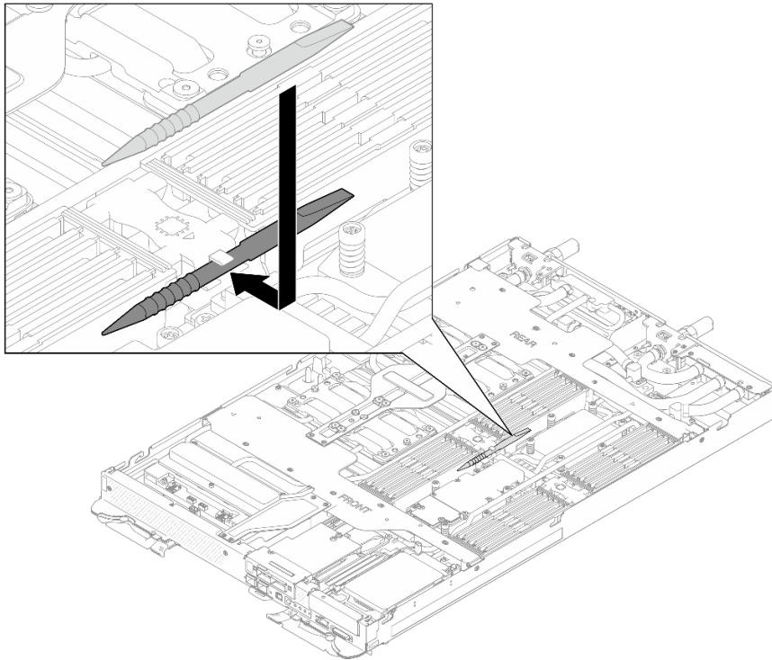
Figura 86. Herramienta del módulo de memoria
