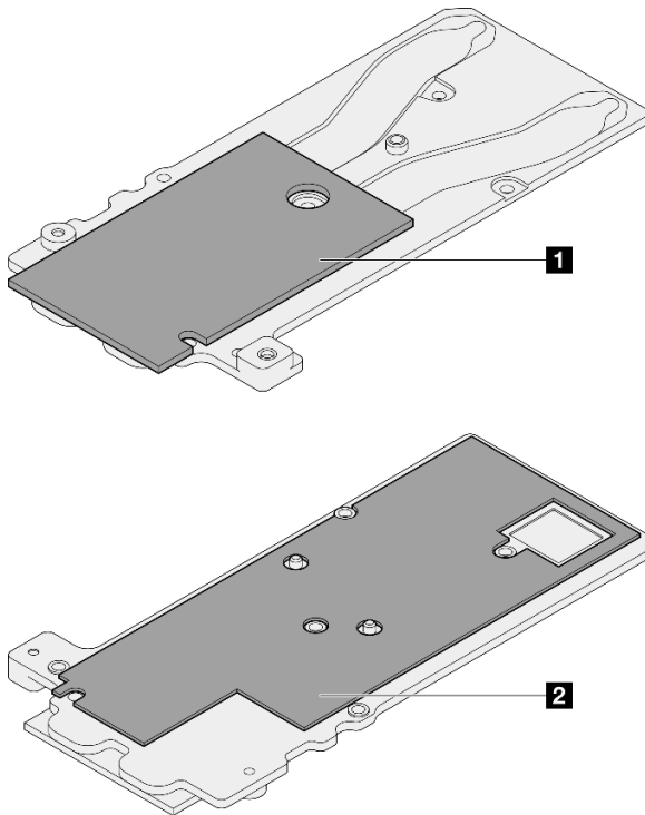
Figura 238. Sustitución de las almohadillas de masilla de la placa de conducción del módulo OSFP
