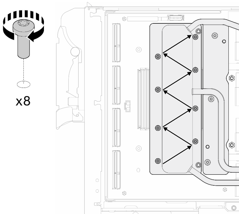
Figura 347. Instalación del tornillo de la tarjeta de red
