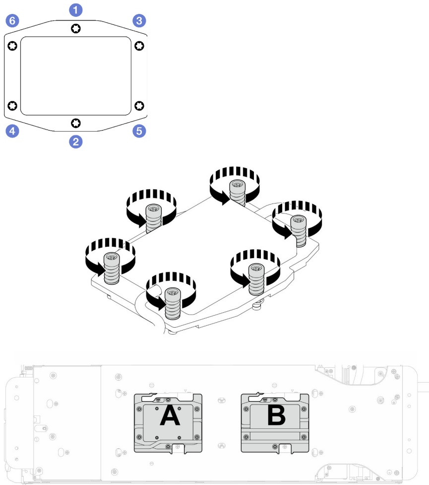
Figura 263. Instalación de la placa de frío del procesador
