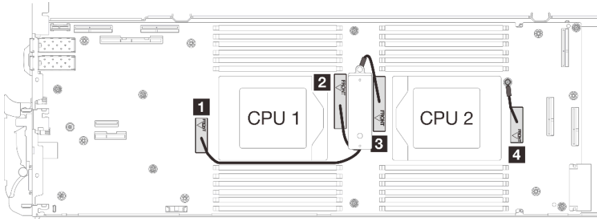
Figura 292. Disposición de los cables para los compartimientos protectores
