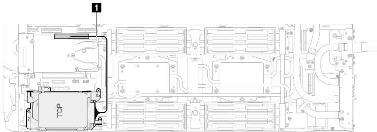
Figura 106. Conexión de los cables del compartimiento de la unidad
