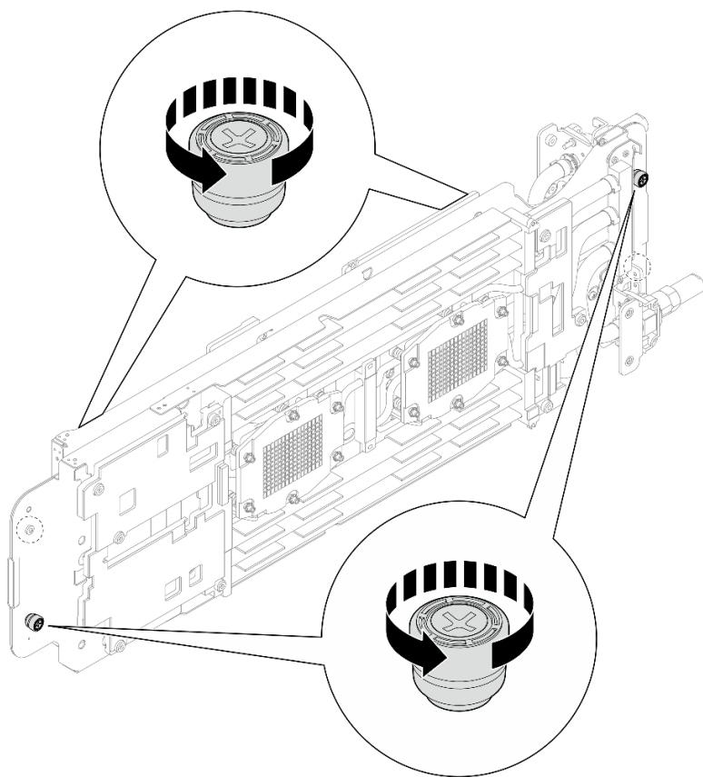
Figura 42. Soltar los tornillos ajustables cautivos del transportador del bucle de agua
