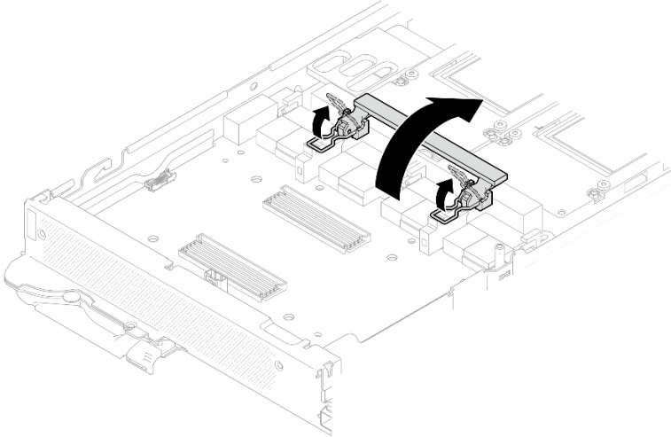
Figura 315. Giro de clips de sujeción y de las manijas de la placa de la GPU
