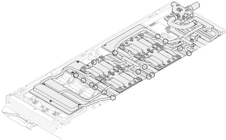
Figura 19. Muecas para soltar las placas de frío de la GPU
