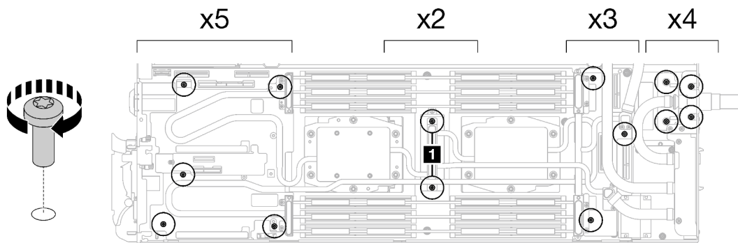
Figura 265. Instalación de los tornillos y tornillos de conexión rápida del bucle de agua
