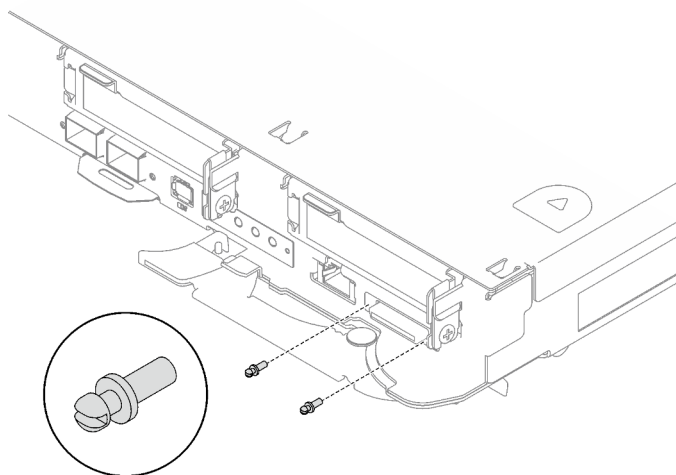
Figura 308. Instalación de los tornillos KVM
