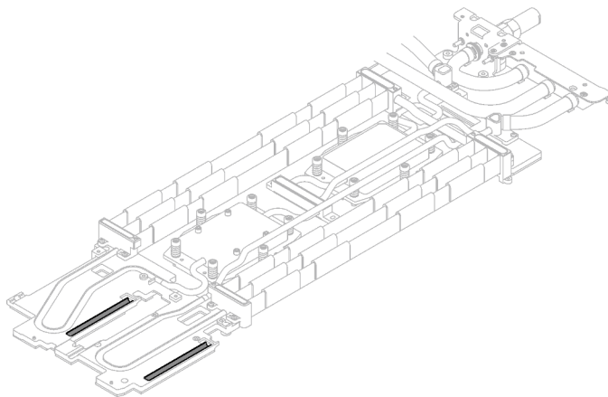
Figura 228. Almohadillas de espacio del bucle de agua (parte superior)
