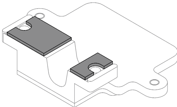
Figura 147. Almohadillas de masilla en la placa de frío de la placa posterior M.2 (parte inferior)
