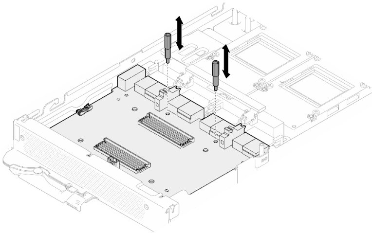
Figura 367. Extracción de los aisladores de la placa del transportador
