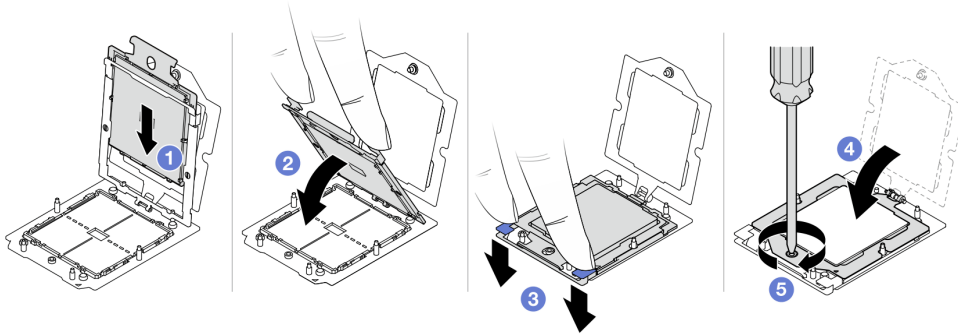
Figura 224. Instalación de un procesador
