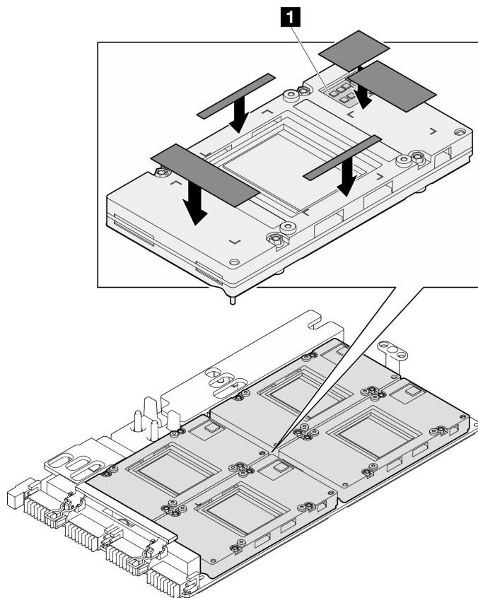
Figura 342. Sustitución de las almohadillas de masilla de la GPU
