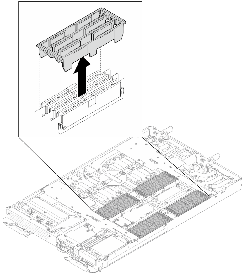
Figura 154. Extracción de la cubierta DIMM
