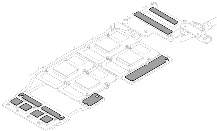
Figura 429. Limpieza de las almohadillas de masilla del bucle de agua
