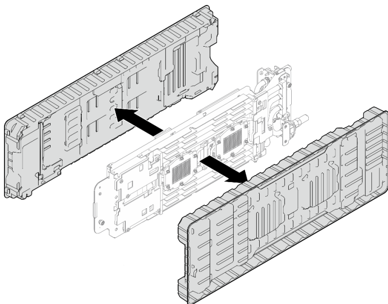
Figura 41. Extracción de las cubiertas de plástico para grasa
