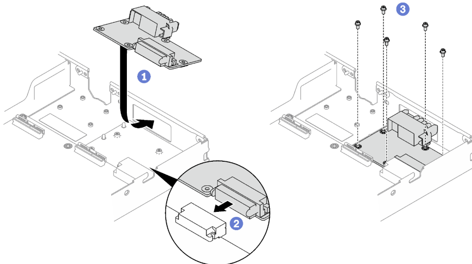
Figura 194. Instalación de la placa de distribución de alimentación
