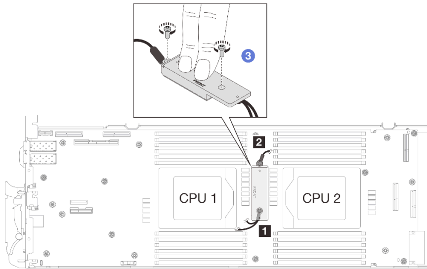
Figura 75. Instalación del cable protector 1/2 y 3
