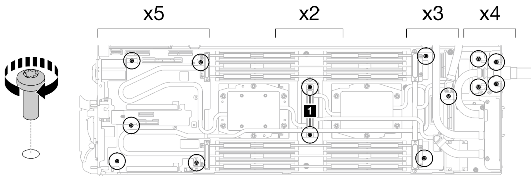
Figura 55. Instalación de los tornillos y tornillos de conexión rápida del bucle de agua
