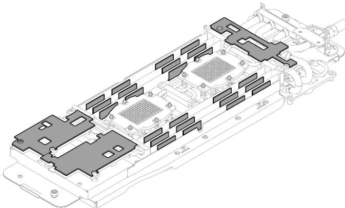
Figura 44. Almohadillas de espacio de la parte inferior del bucle de agua (lado del nodo de cálculo)
