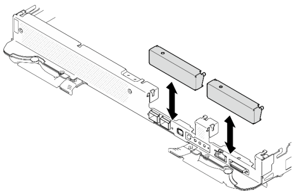
Figura 116. Instalación del relleno vacío del marco biselado
