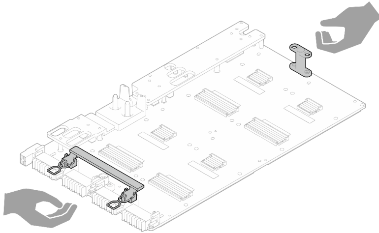
Figura 360. Extracción de la placa de GPU de la caja del paquete
