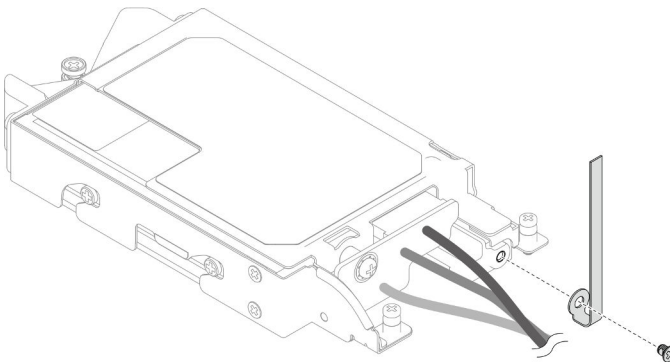
Figura 125. Extracción de la brida de cables
