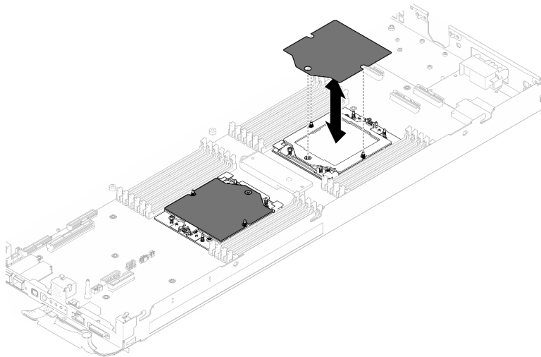
Figura 253. Instalación de la película protectora del zócalo del procesador
