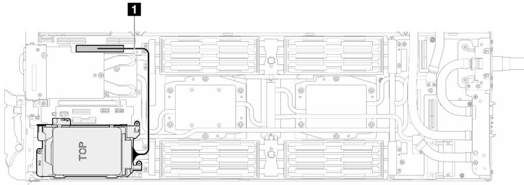
Figura 107. Desconexión del cable de la unidad
