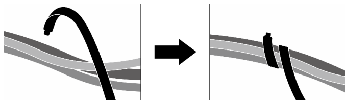
Figura 451. Atado de la brida de cables
