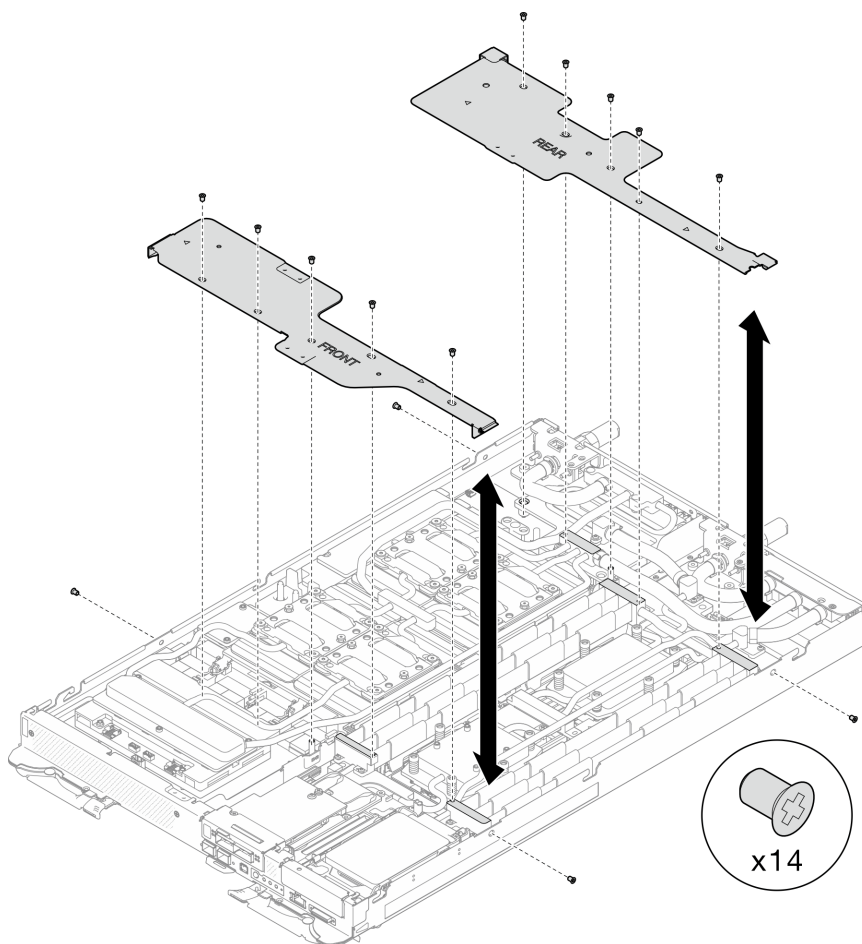
Figura 8. Extracción de las llaves cruzadas frontales y traseras
