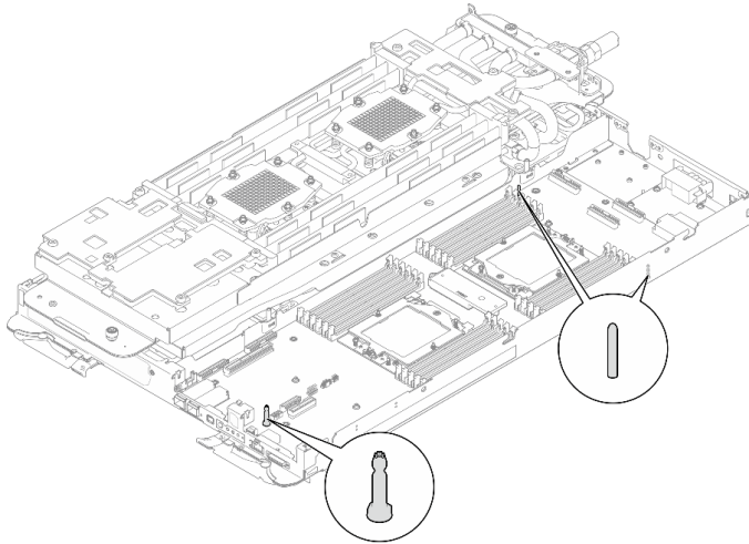
Figura 199. Patillas guía en el nodo de cálculo
