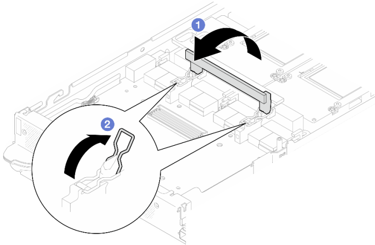
Figura 354. Liberación de la placa del transportador
