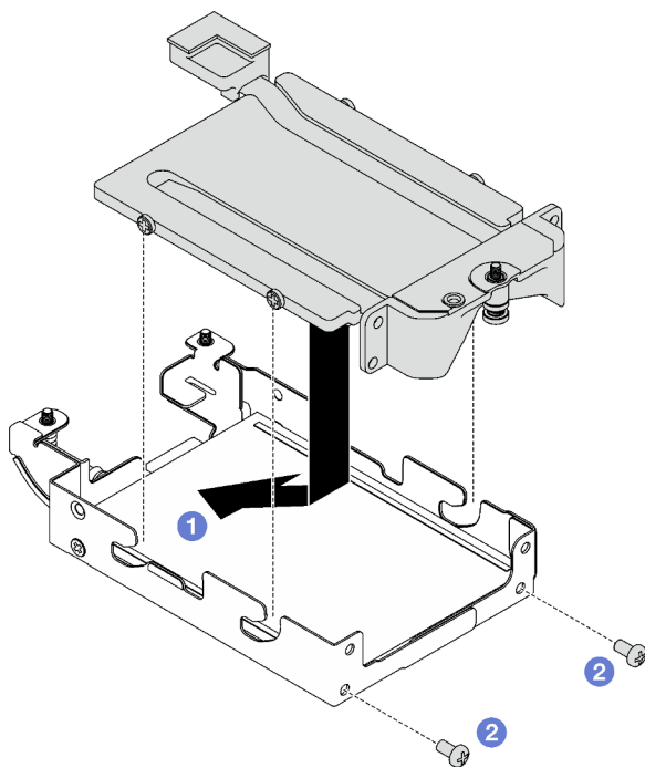
Figura 133. Instalación de la placa de conducción de la unidad E3.s
