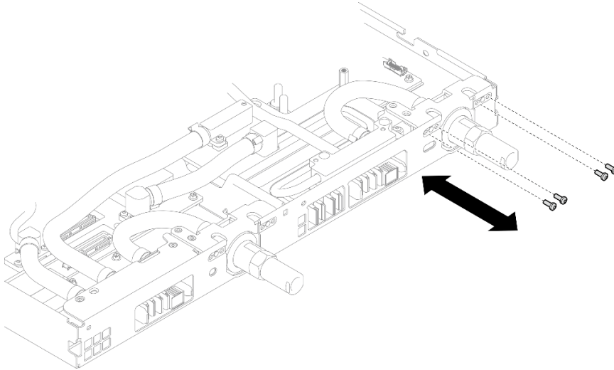
Figura 419. Extracción del tornillo de la conexión rápida (nodo de la GPU)
