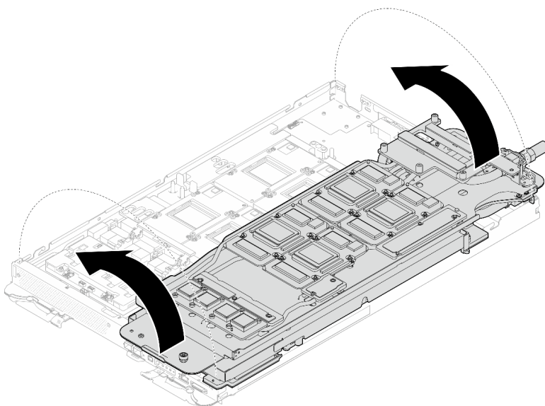
Figura 343. Despliegado del bucle de agua en el nodo de la GPU
