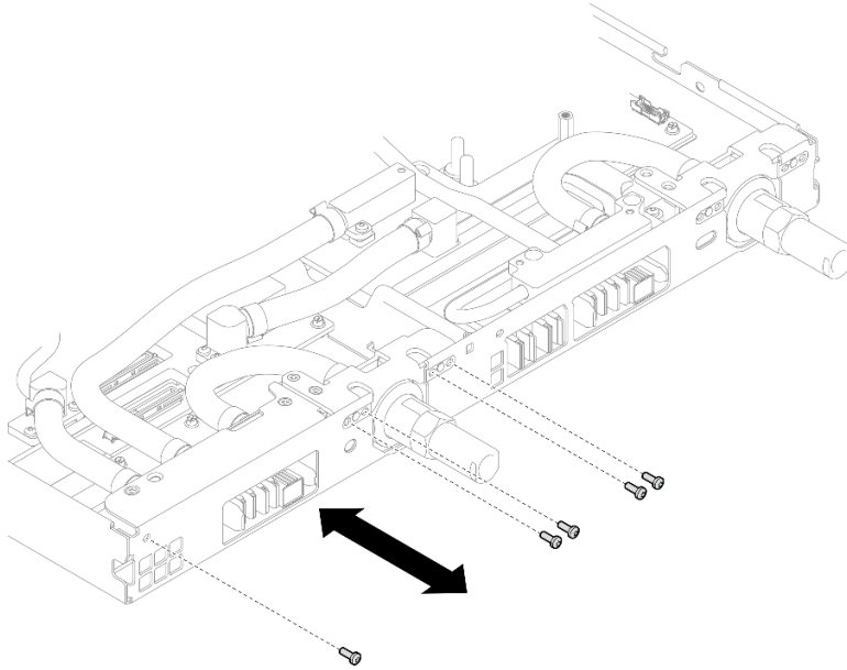
Figura 237. Instalación del tornillo de la conexión rápida (nodo de cálculo)
