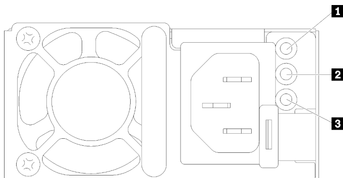
Figura 459. LED de la fuente de alimentación de CA
