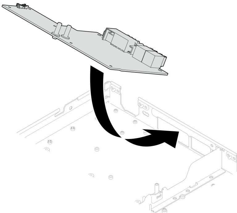
Figura 399. Instalación de la placa de distribución de alimentación de la GPU
