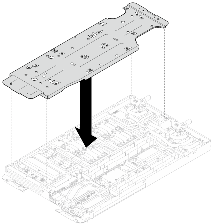
Figura 21. Instalación del transportador del bucle de agua (nodo de la GPU)
