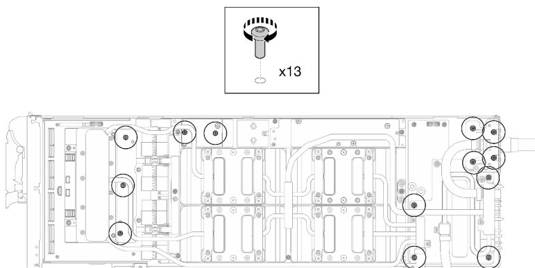
Figura 410. Instalación de los tornillos Torx T10 del bucle de agua (nodo de la GPU)
