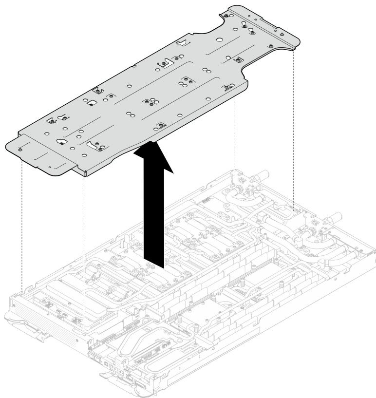
Figura 406. Extracción del transportador del bucle de agua (nodo de la GPU)
