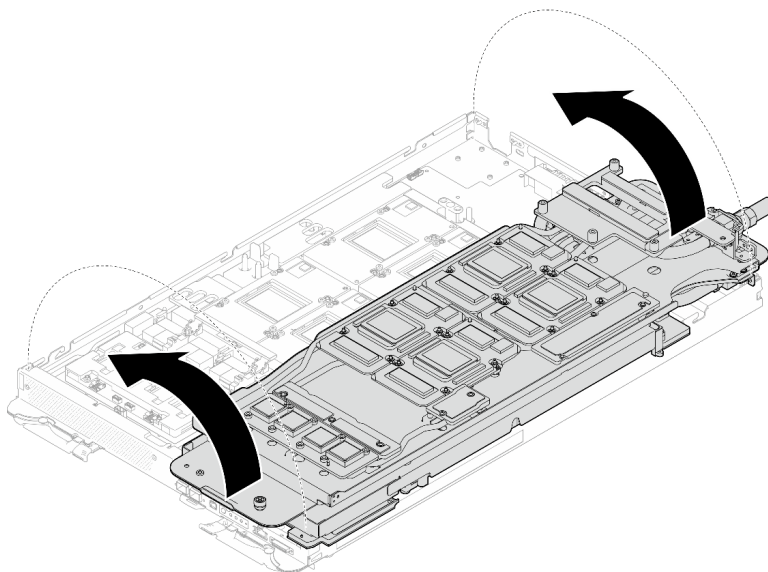
Figura 404. Despliegado del bucle de agua en el nodo de la GPU
