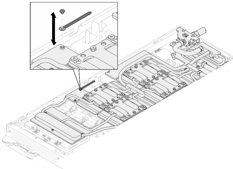
Figura 12. Extracción de la brida de cables
