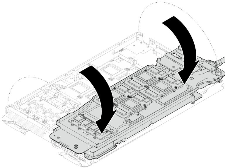
Figura 393. Plegado del bucle de agua del lado del nodo de la GPU en el bucle de agua del lado del nodo de cálculo
