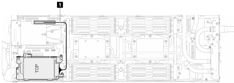
Figura 180. Conexión del cable de la unidad
