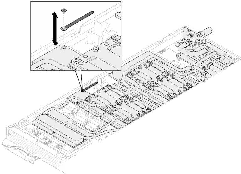
Figura 412. Instalación de la brida de cables
