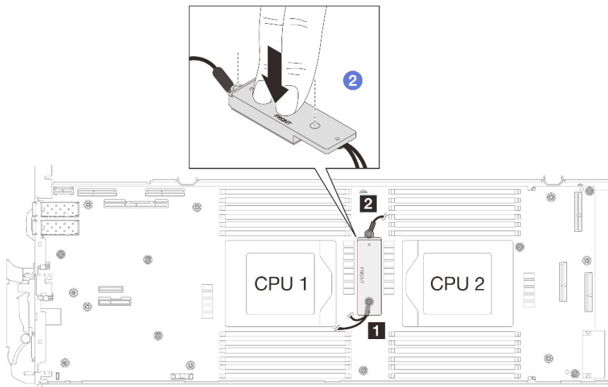
Figura 298. Presión en la placa de conducción de VR
