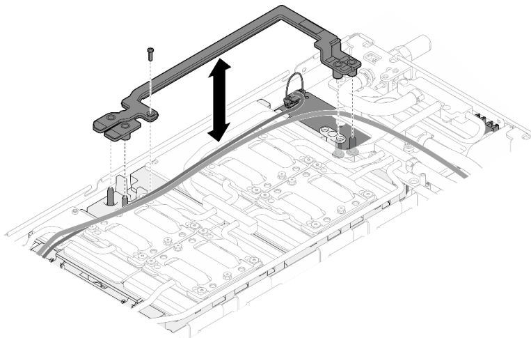
Figura 311. Instalación de la barra de bus
