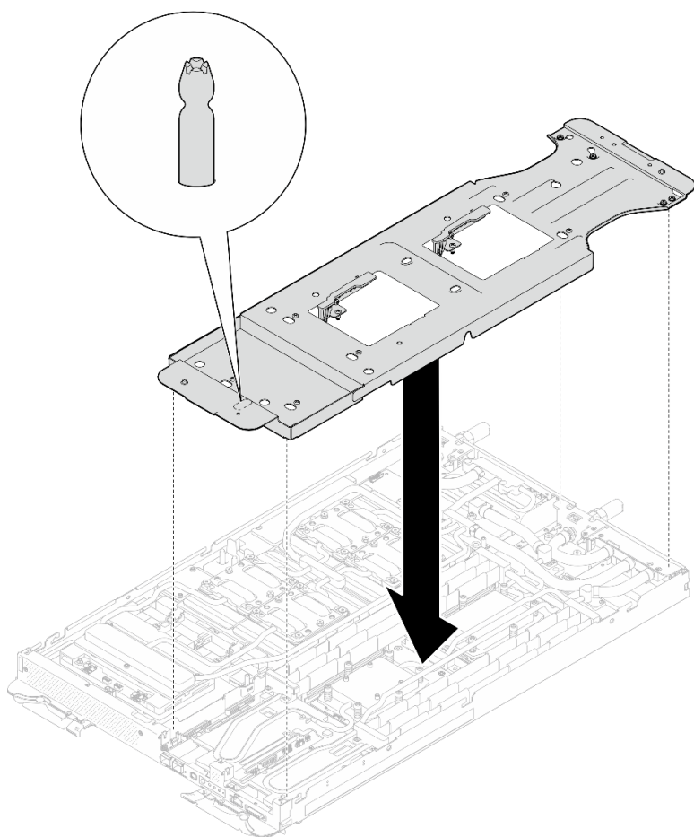
Figura 218. Instalación del transportador del bucle de agua (nodo de cálculo)
