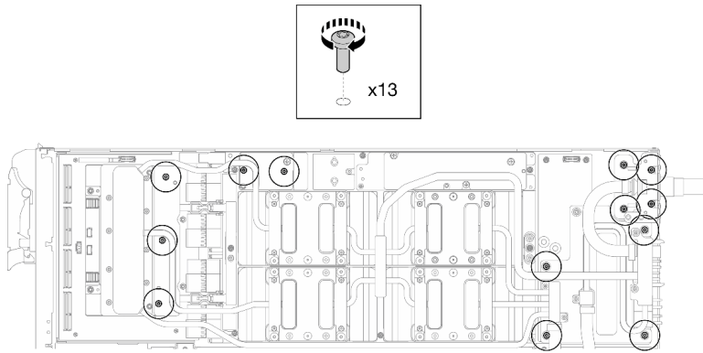
Figura 349. Instalación de los tornillos Torx T10 del bucle de agua (nodo de la GPU)
