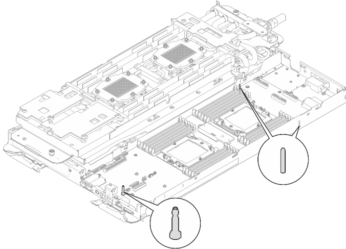
Figura 259. Patillas guía en el nodo de cálculo
