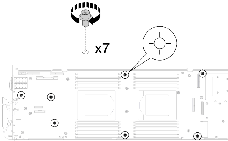
Figura 303. Instalación de los tornillos de la placa del sistema
