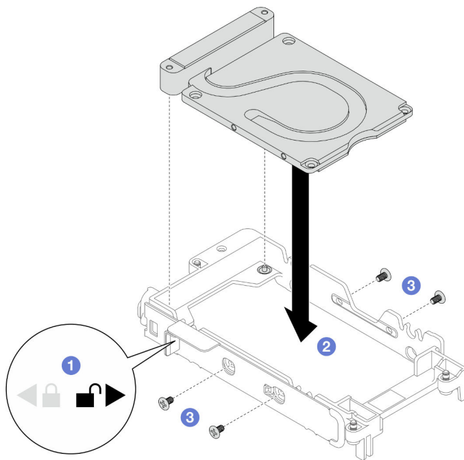
Figura 113. Instalación de la placa de conducción
