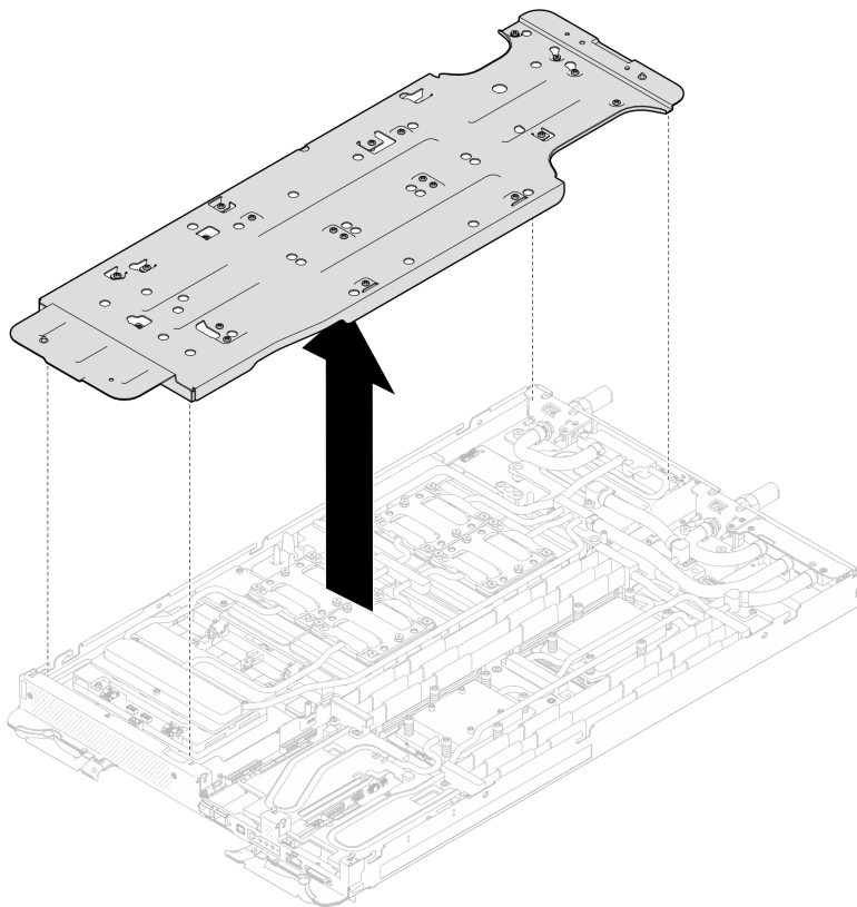
Figura 439. Extracción del transportador del bucle de agua (nodo de la GPU)
