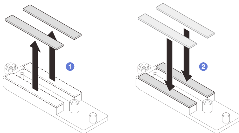
Figura 305. Sustitución de las almohadillas de masilla de la placa de conducción de VR
