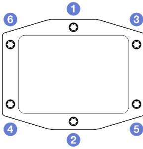
Figura 187. Etiqueta de la placa de frío del procesador
