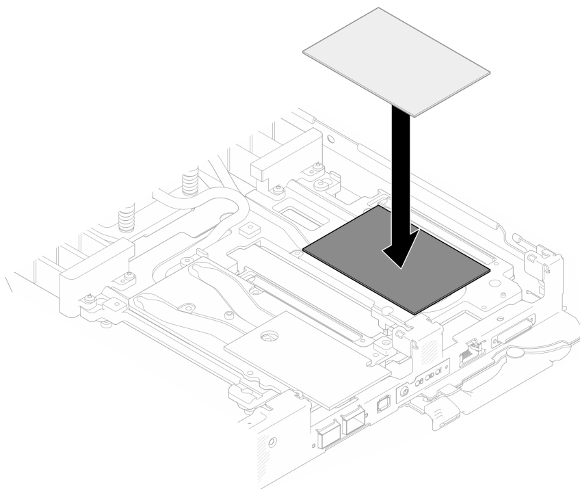
Figura 139. Sustituir la almohadilla de espacio
