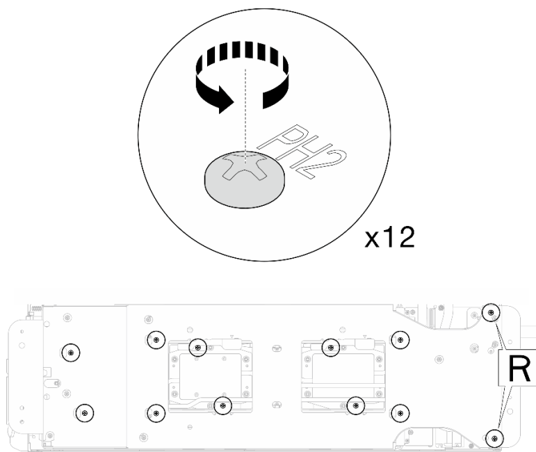
Figura 35. Instalación de los tornillos del transportador del bucle de agua (nodo de cálculo)
