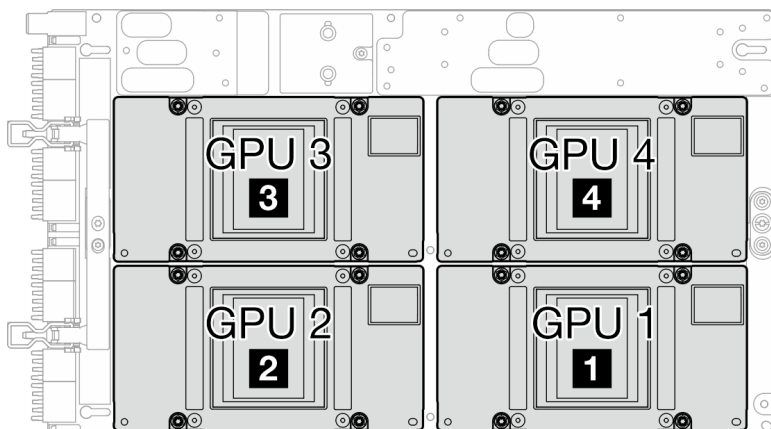
Figura 337. Numeración de la GPU
