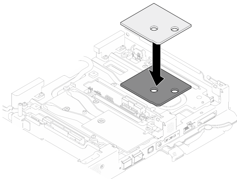
Figura 118. Sustituir la almohadilla de espacio
