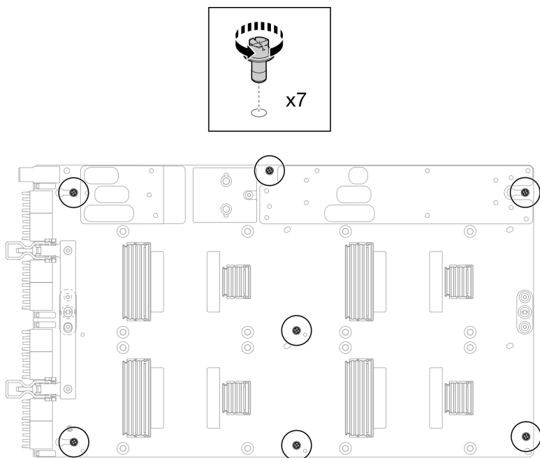
Figura 356. Extracción de los tornillos M3 de la placa de la GPU
