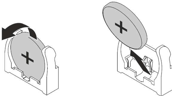
Figura 80. Extracción de la batería CMOS
