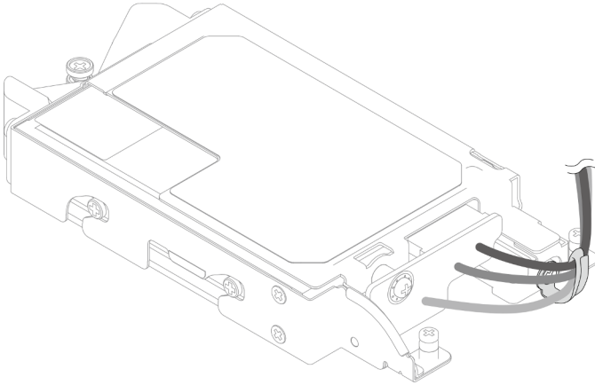
Figura 124. Soltar los cables de la brida de cables
