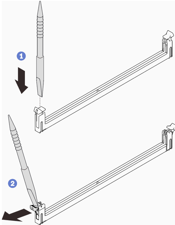
Figura 155. Extracción del módulo de memoria
