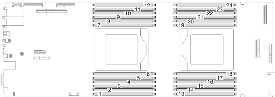
Figura 152. Ubicación del conector del módulo de memoria
