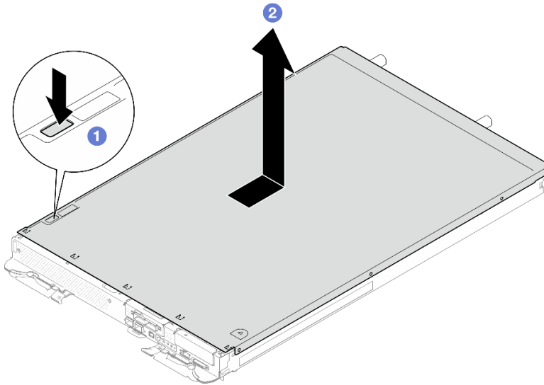
Figura 5. Extracción de la cubierta de bandeja
