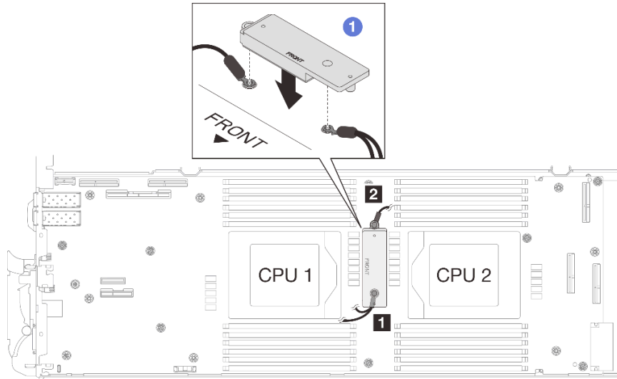
Figura 297. Alineación de la placa de conducción de VR, cables protectores y orificios para los tornillos de la placa del sistema
