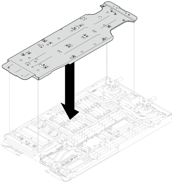
Figura 391. Instalación del transportador del bucle de agua (nodo de la GPU)
