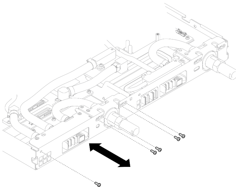
Figura 213. Extracción del tornillo de la conexión rápida (nodo de cálculo)
