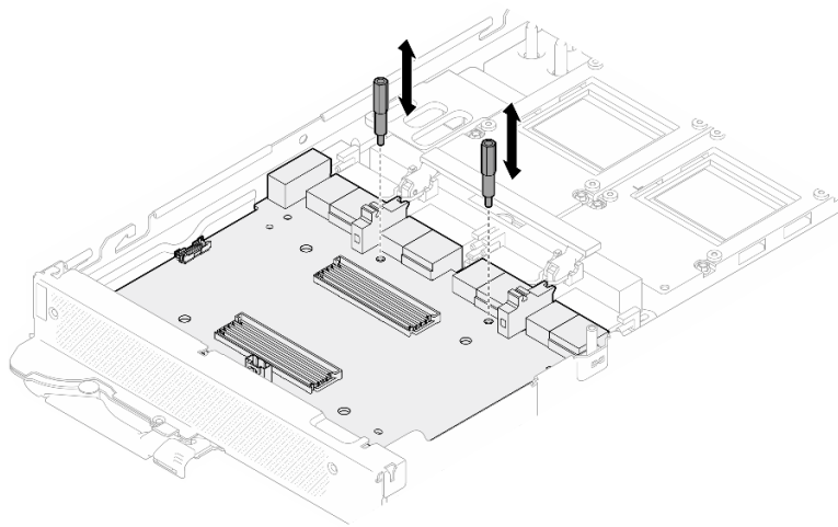
Figura 366. Instalación de los aisladores de la placa del transportador
