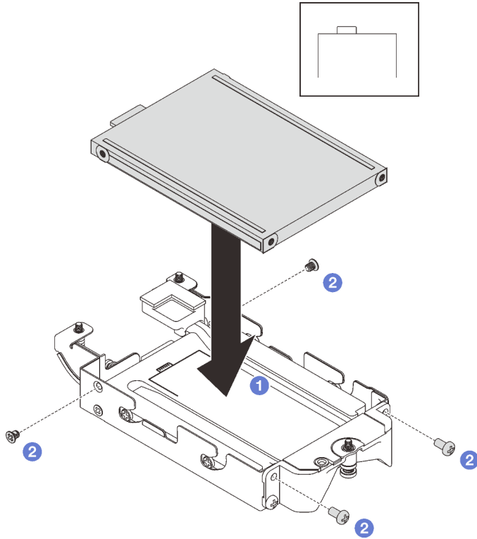
Figura 134. Instalación de la unidad E3.s inferior
