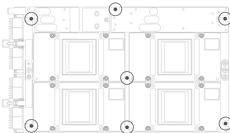
Figura 375. Instalación de los tornillos M3 en el conjunto de la placa de la GPU
