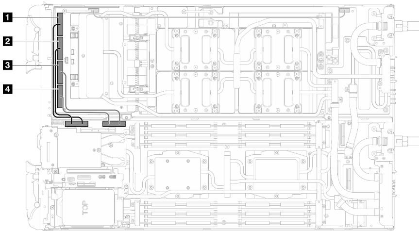
Figura 178. Configuración de un procesador - Conexión de todos los cables MCIO a la placa del transportador
