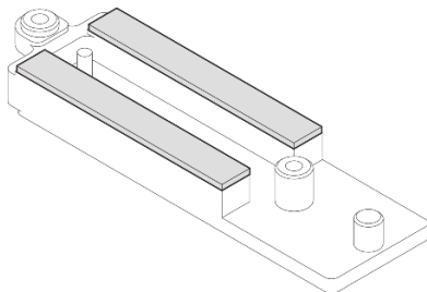
Figura 77. Las almohadillas de masilla se encuentran en la parte inferior de la placa de conducción del VR
