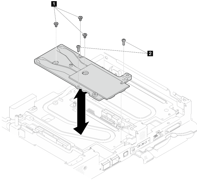
Figura 239. Instalación de la placa de conducción del Módulo OSFP
