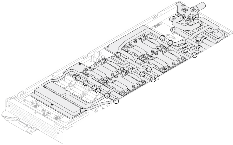
Figura 389. Muecas para soltar las placas de frío de la GPU
