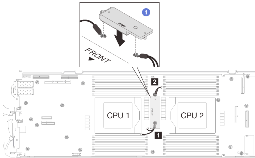
Figura 73. Alineación de la placa de conducción de VR, cables protectores y orificios para los tornillos de la placa del sistema
