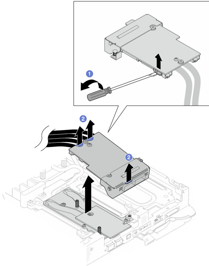
Figura 172. Extracción del Módulo OSFP
