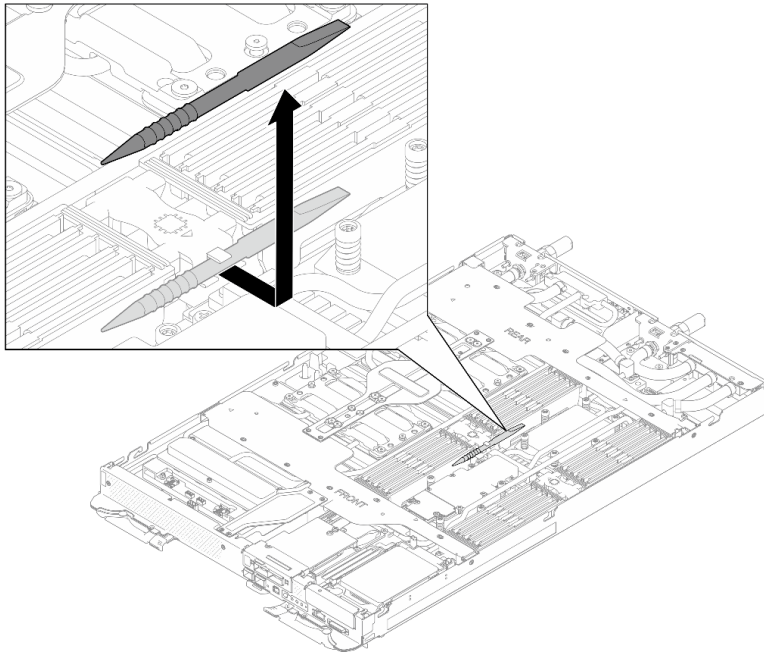
Figura 83. Extracción de la herramienta del módulo de memoria
