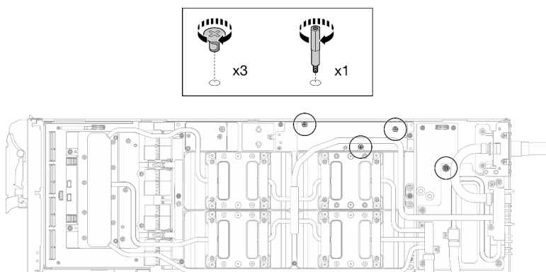
Figura 411. Instalación de los tornillos hexagonal y PH1 del bucle de agua (nodo de la GPU)
