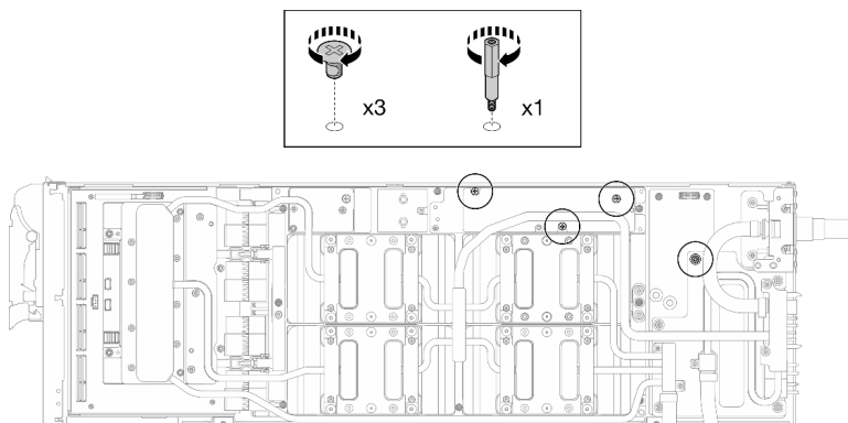
Figura 350. Instalación de los tornillos hexagonal y PH1 del bucle de agua (nodo de la GPU)
