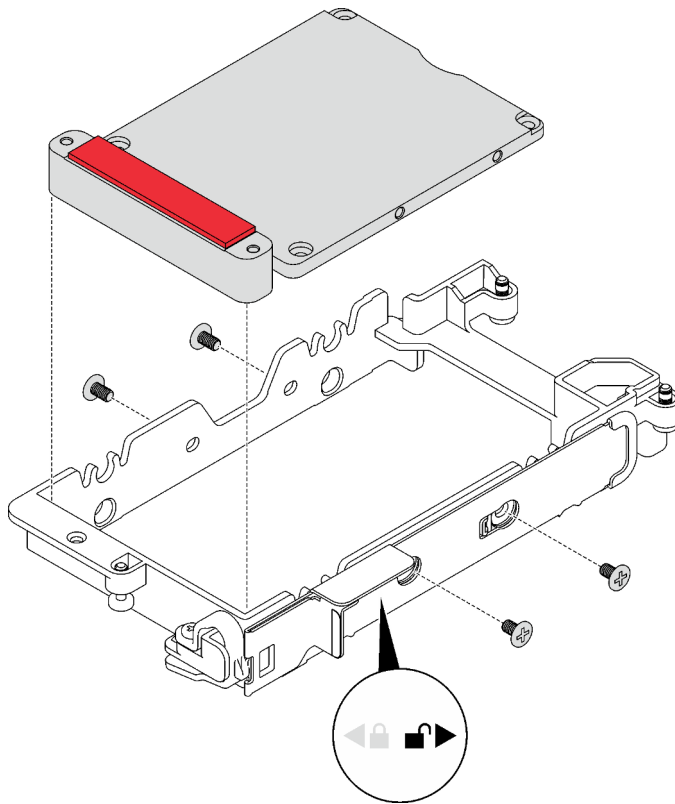
Figura 94. Extracción de la placa de conducción
