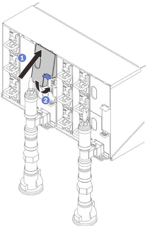
Figura 467. Instalación de protecciones EMC superiores
