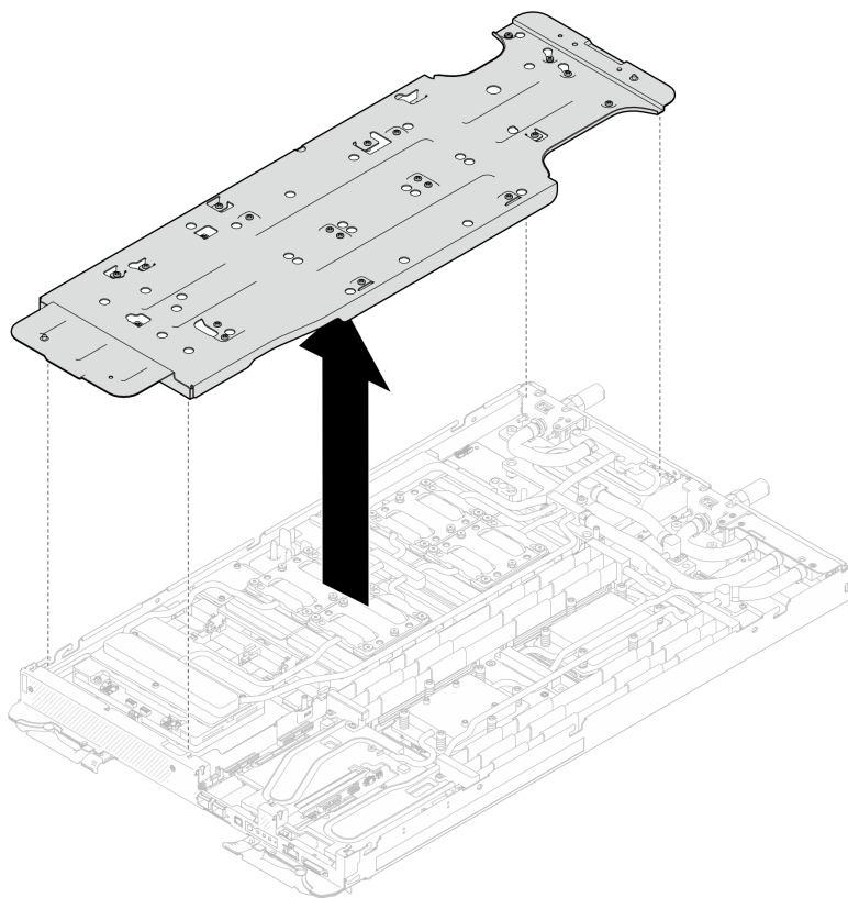
Figura 345. Extracción del transportador del bucle de agua (nodo de la GPU)
