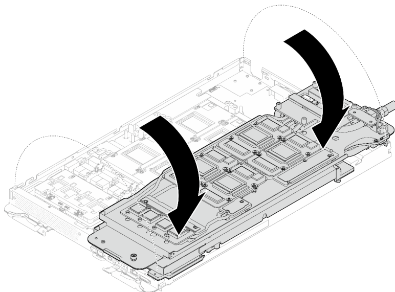
Figura 333. Plegado del bucle de agua del lado del nodo de la GPU en el bucle de agua del lado del nodo de cálculo
