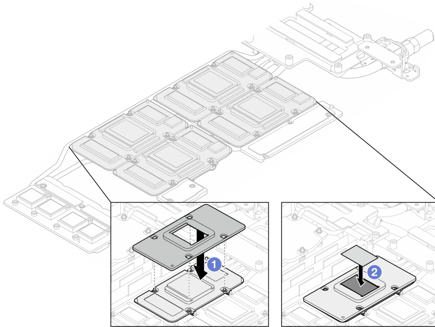
Figura 46. Sustitución del PCM de la placa de frío del bucle de agua de la GPU (nodo de GPU)
