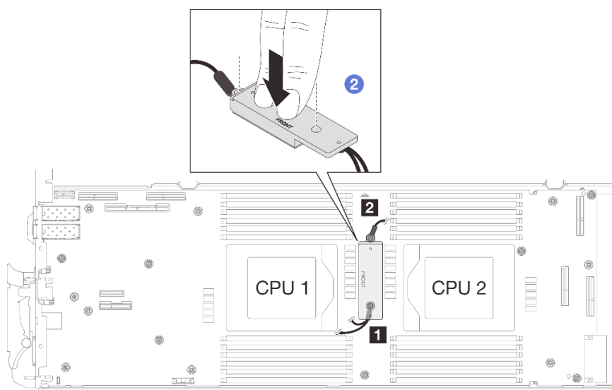
Figura 281. Presión en la placa de conducción de VR
