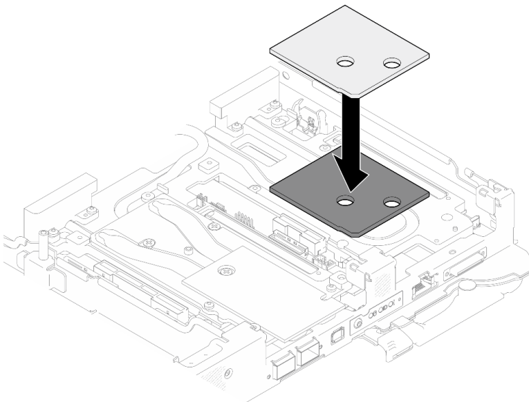
Figura 103. Sustituir la almohadilla de espacio
