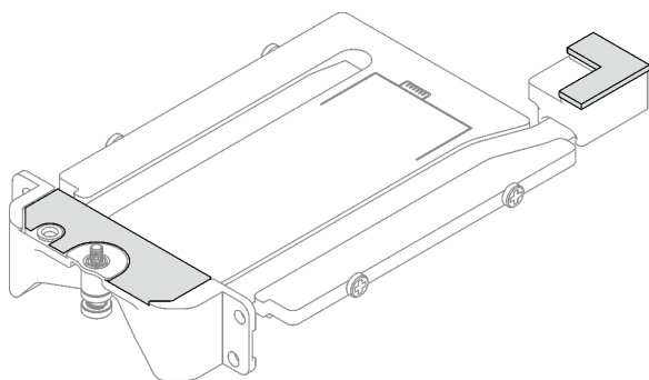
Figura 132. Sustitución de las almohadillas de masilla de la placa de conducción
