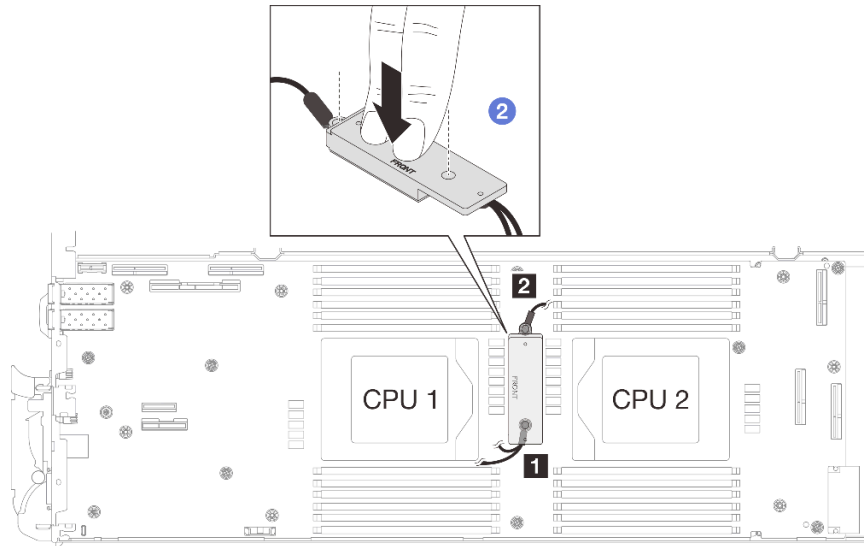
Figura 74. Presión en la placa de conducción de VR
