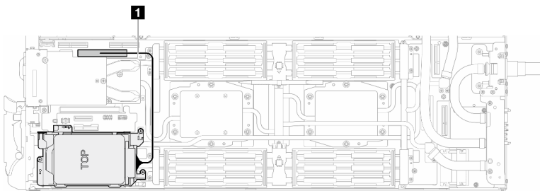
Figura 87. Desconexión del cable de la unidad
