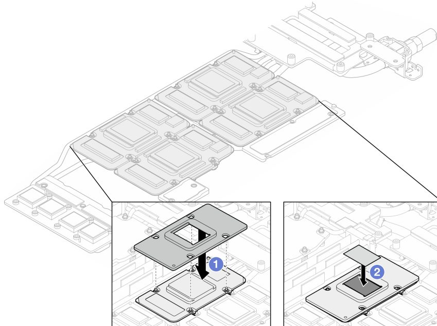
Figura 340. Sustitución del PCM de la placa de frío del bucle de agua de la GPU (nodo de GPU)
