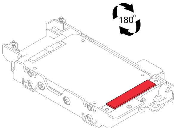
Figura 101. Ubicación de las almohadillas de espacio
