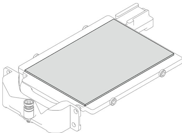
Figura 131. Sustitución de la almohadilla de espacio de la placa de conducción
