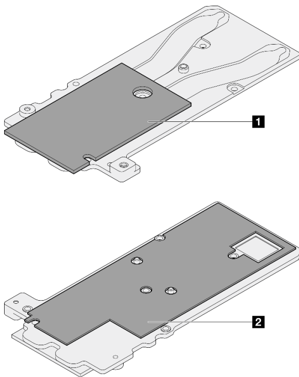
Figura 207. Sustitución de las almohadillas de masilla de la placa de conducción del módulo OSFP
