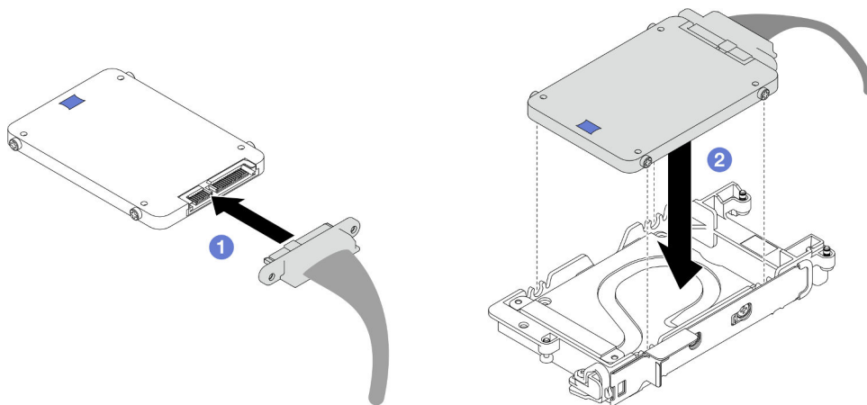
Figura 114. Instalación de la unidad inferior
