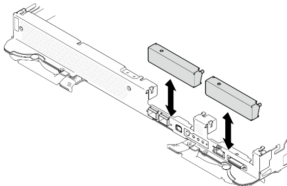
Figura 90. Extracción del relleno vacío del marco biselado
