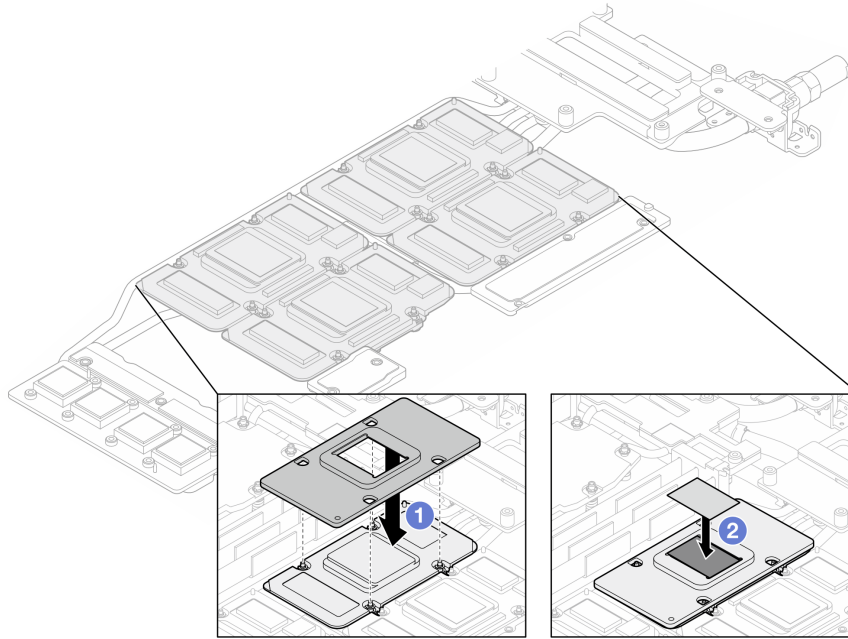
Figura 401. Sustitución del PCM de la placa de frío del bucle de agua de la GPU (nodo de GPU)
