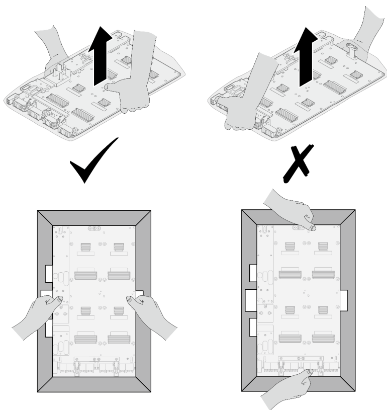
Figura 359. Extracción de la placa de GPU de la caja del paquete
