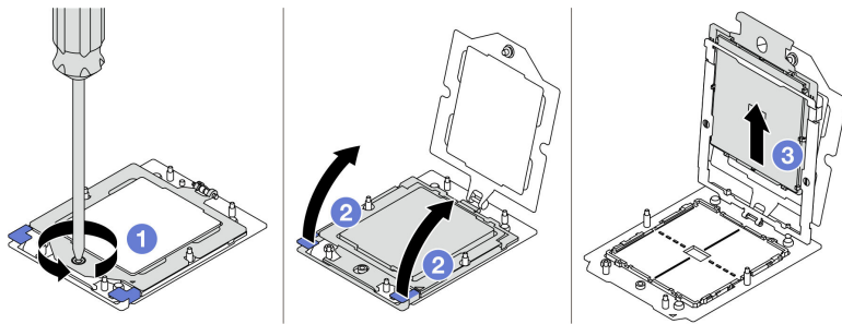
Figura 222. Extracción de un procesador
