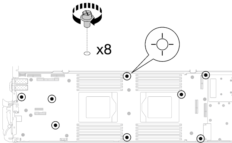
Figura 272. Extracción de los tornillos de la placa del sistema
