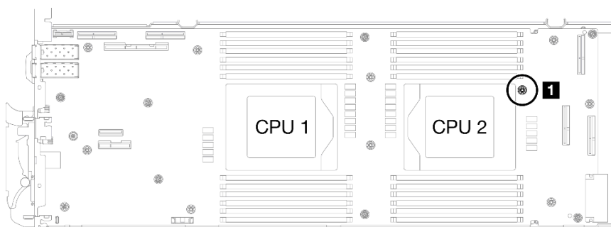
Figura 283. Ubicación del orificio de tornillo del cable protector 4
