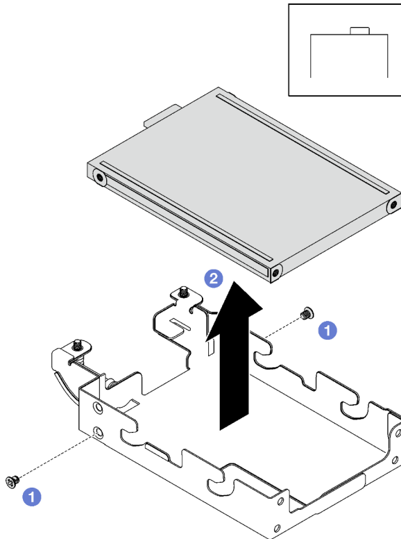
Figura 129. Extracción de la unidad E3.s superior
