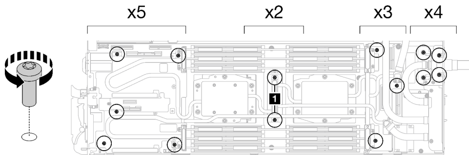
Figura 245. Extracción del tornillo del bucle de agua
