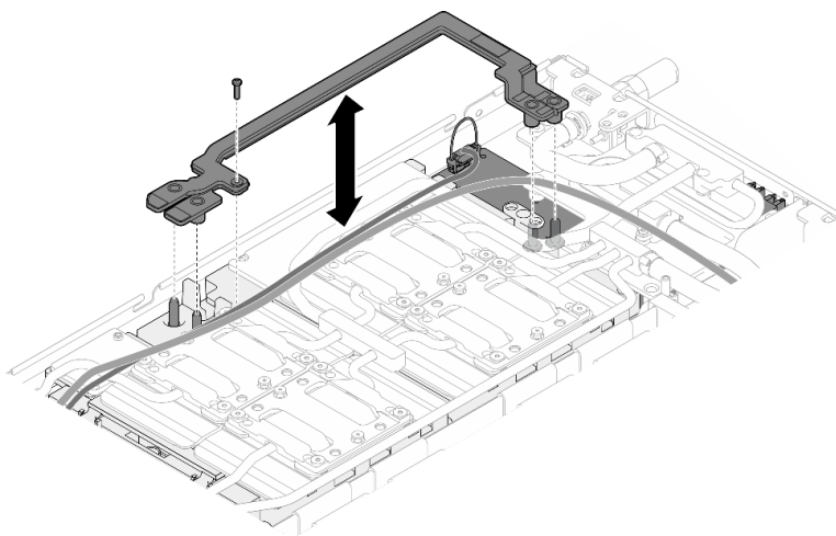
Figura 309. Extracción de la barra de bus
