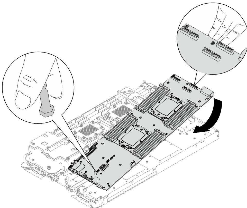
Figura 296. Instalación de la placa del sistema
