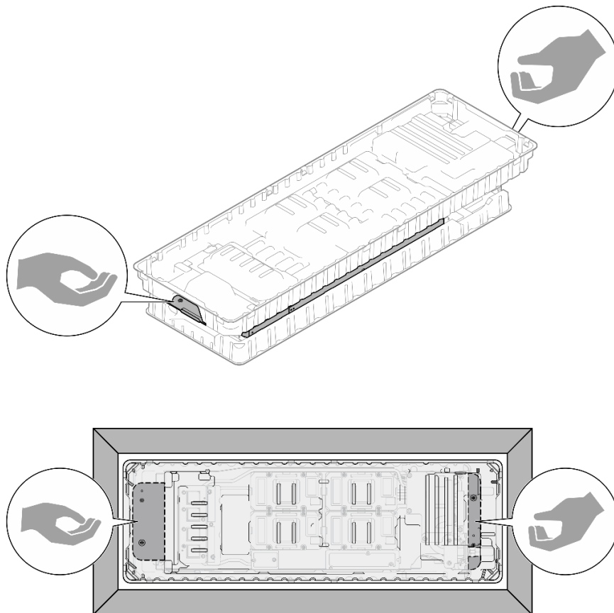
Figura 40. Puntos de contacto al extraer el bucle de agua de la caja de embalaje
