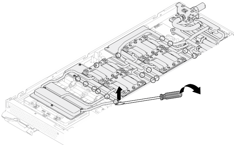
Figura 424. Liberación de la placa de frío de la GPU desde la GPU
