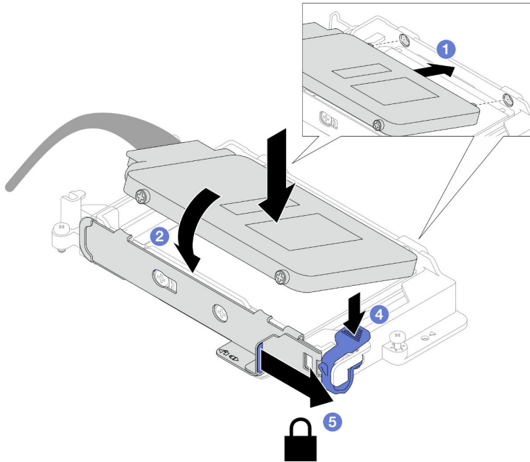
Figura 115. Instalación de la unidad superior
