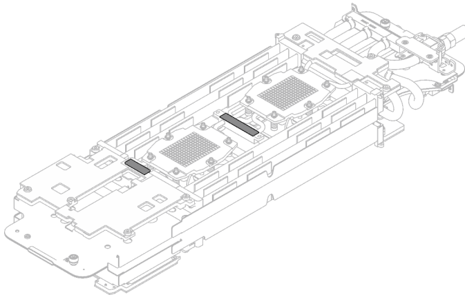
Figura 43. Almohadillas de masilla de la parte inferior del bucle de agua (lado del nodo de cálculo)
