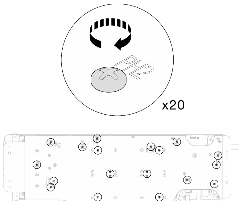
Figura 332. Extracción del tornillo del bucle de agua y del tornillo de conexión rápida (nodo de la GPU)
