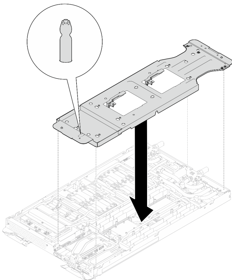
Figura 34. Instalación del transportador del bucle de agua (nodo de cálculo)
