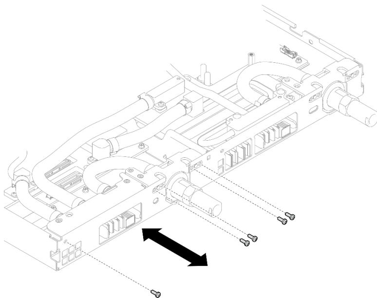
Figura 206. Instalación del tornillo de la conexión rápida (nodo de cálculo)
