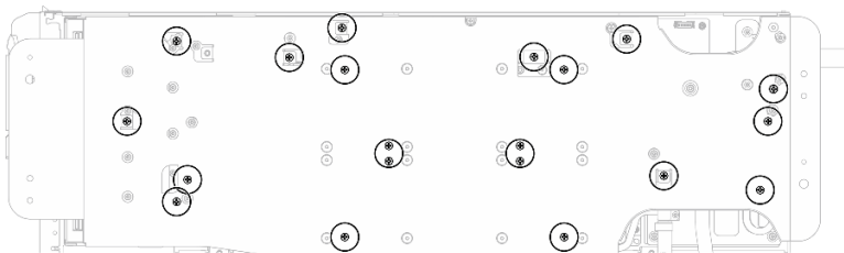
Figura 426. Extracción del tornillo del bucle de agua y del tornillo de conexión rápida (nodo de la GPU)
