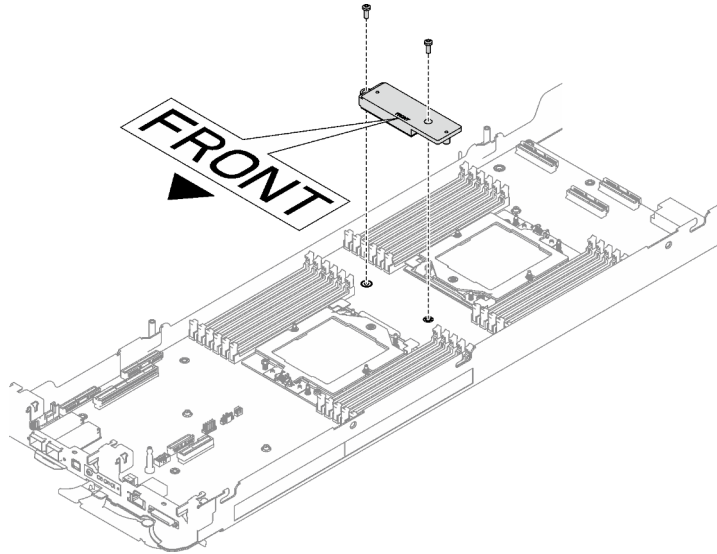
Figura 76. Extracción de la placa de conducción del VR
