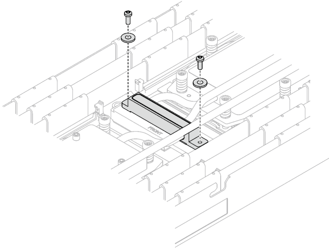
Figura 204. Tornillos de la placa de frío del VR con arandela
