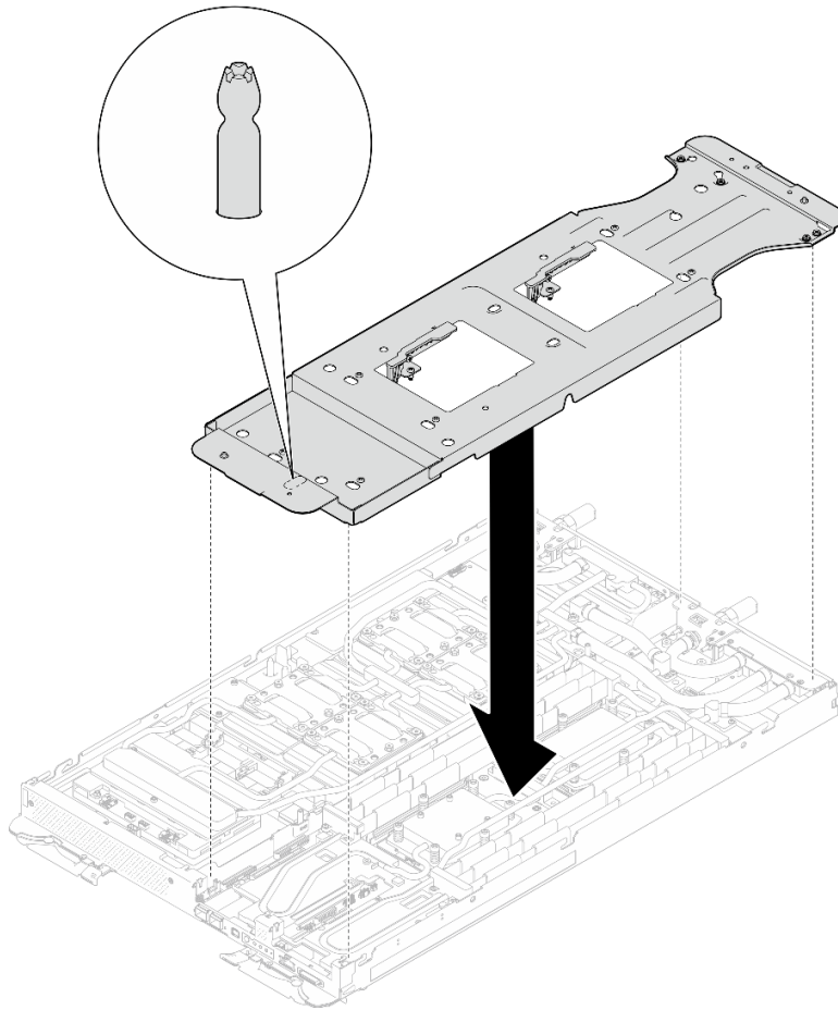
그림 248. 워터 루프 캐리어 설치(컴퓨팅 노드)
