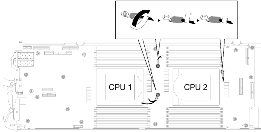
그림 285. 차폐 케이블에 레이블 감기
