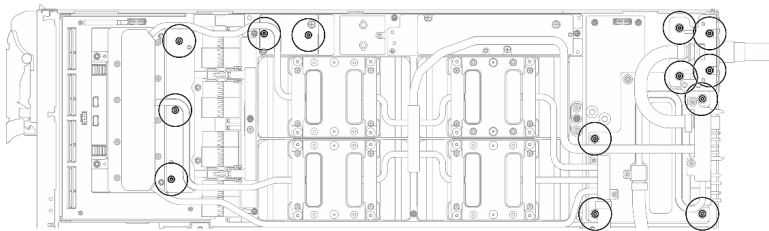
그림 324. 워터 루프 Torx T10 나사 제거(GPU 노드)
