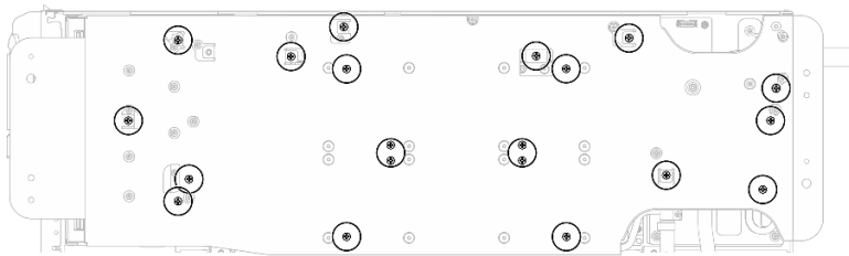
그림 438. 워터 루프 나사 및 퀵 커넥트 나사 설치(GPU 노드)
