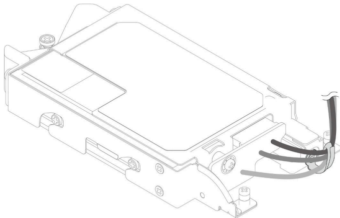
그림 137. 케이블 타이로 케이블 묶기
