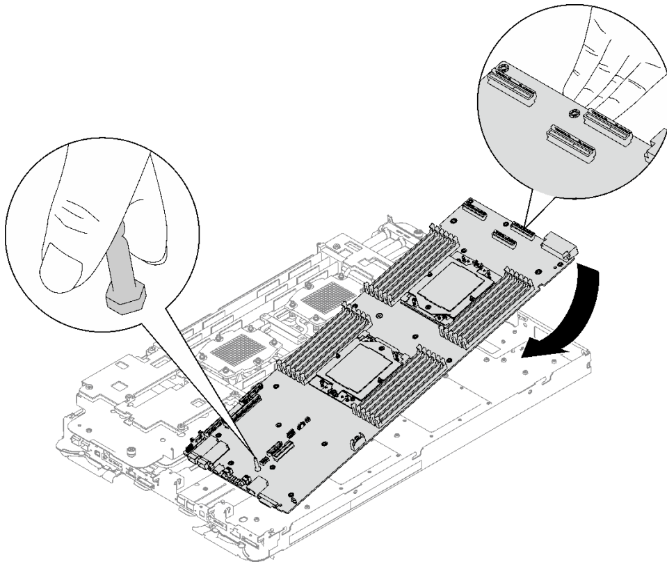
그림 296. 시스템 보드 설치
