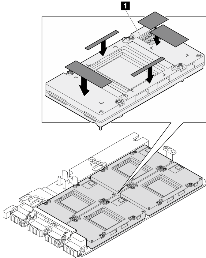
그림 342. GPU 퍼티 패드 교체
