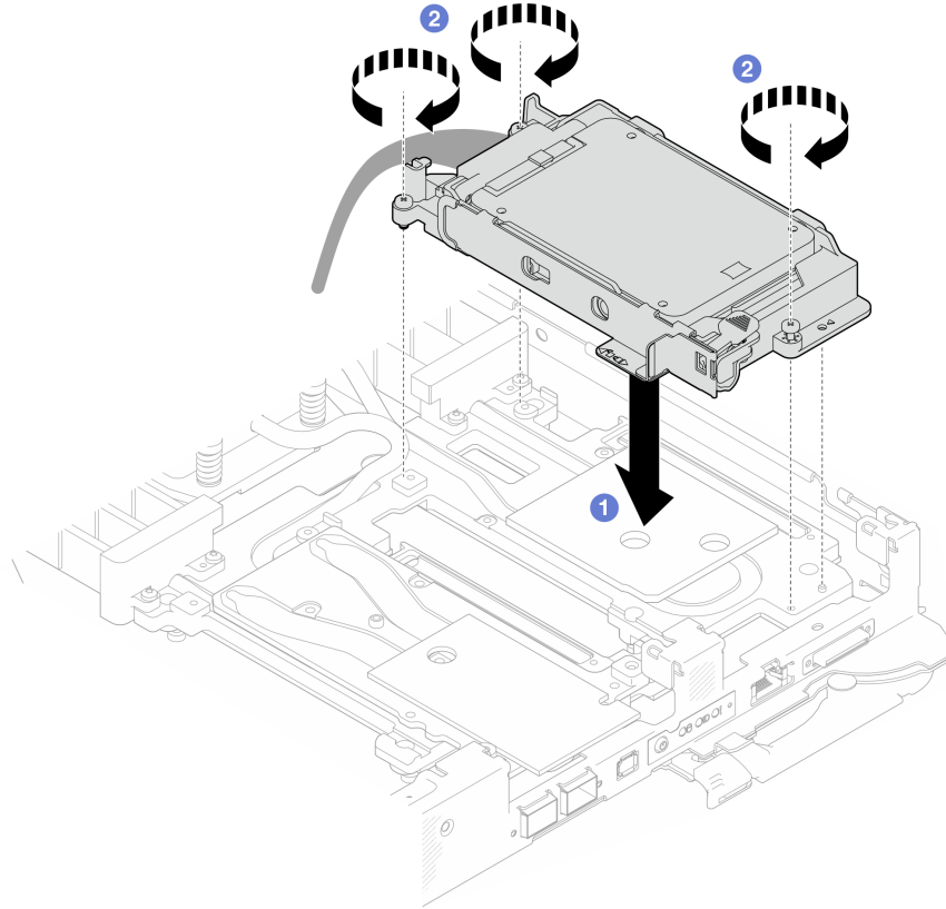
그림 119. 7mm NVMe 드라이브 케이지 어셈블리 설치
