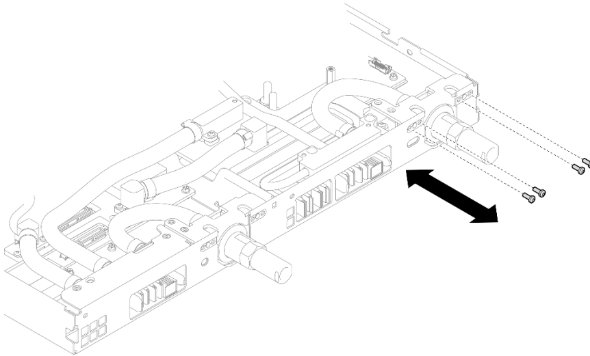
그림 15. 퀵 커넥트 나사 제거(GPU 노드)
