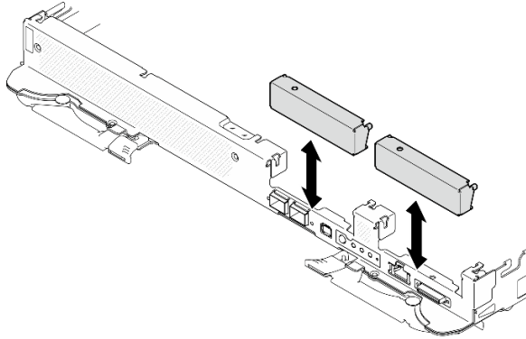
그림 123. 빈 베젤 필러 제거
