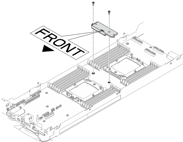
그림 306. VR 전도판 설치
