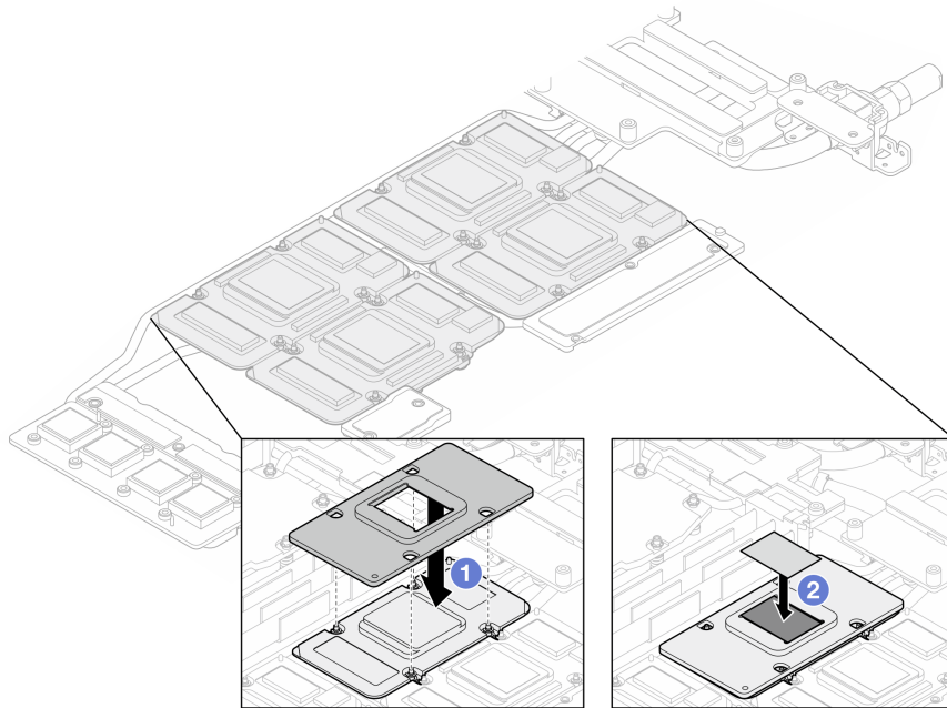
그림 340. 워터 루프 GPU 냉각판 PCM 교체(GPU 노드)
