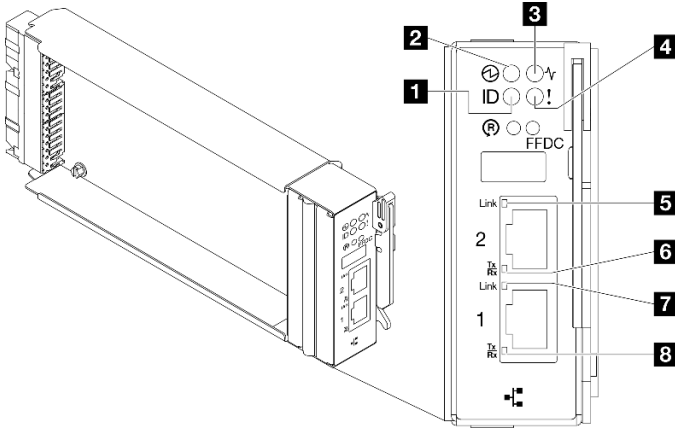
그림 458. SMM2 LED
