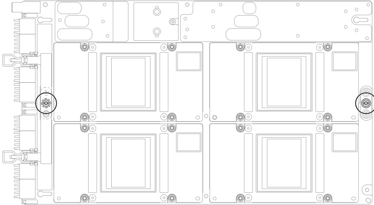
그림 371. GPU 보드 어셈블리 T15 나사 제거
