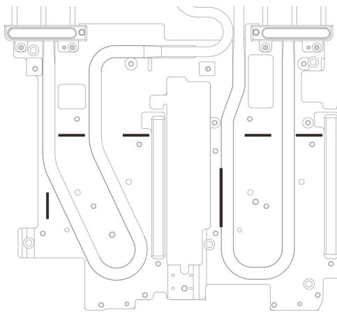
그림 117. 갭 패드를 맞추기 위한 워터 루프의 표시
