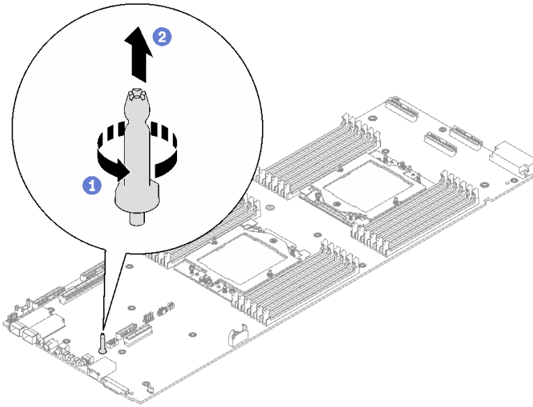
그림 274. 가이드 핀 제거
