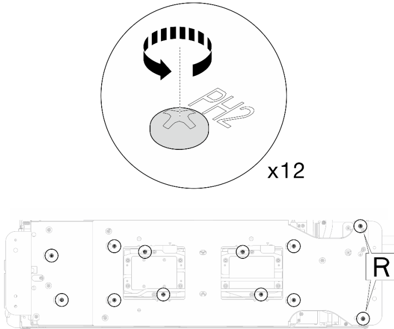
그림 232. 워터 루프 캐리어 나사 풀기
