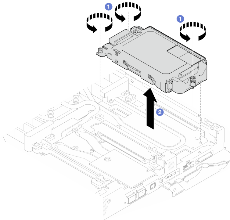
그림 122. E3.S 드라이브 케이징 어셈블리 제거
