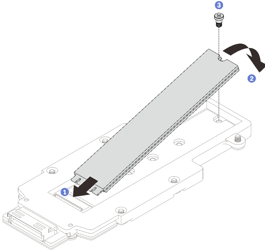
그림 146. M.2 드라이브 설치
