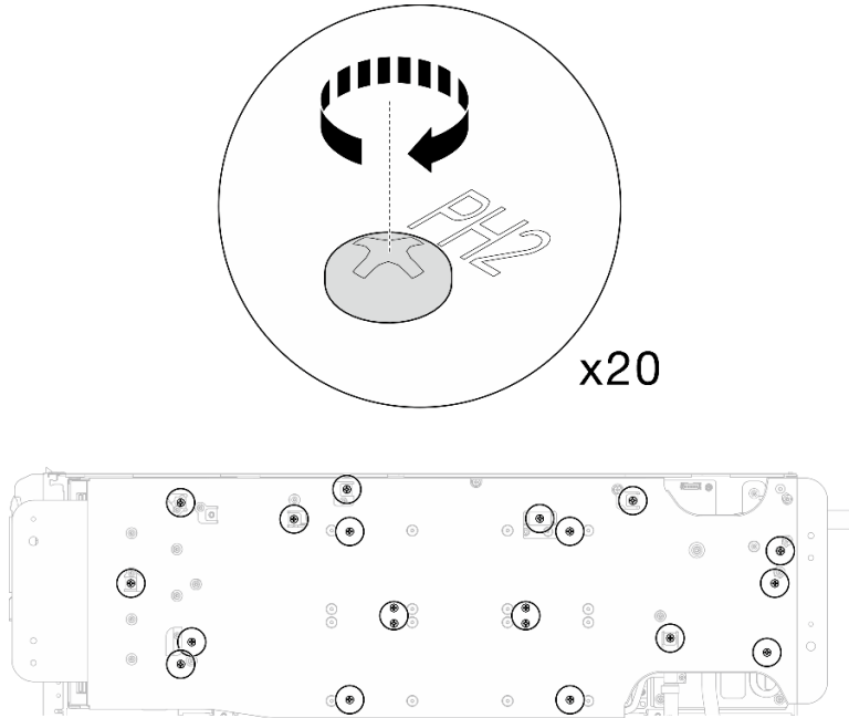
그림 392. 워터 루프 나사 및 빠른 연결 나사 제거(GPU 노드)
