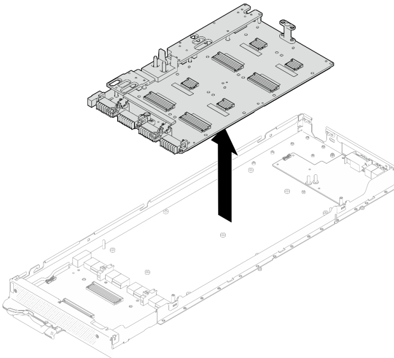
그림 358. GPU 보드 제거
