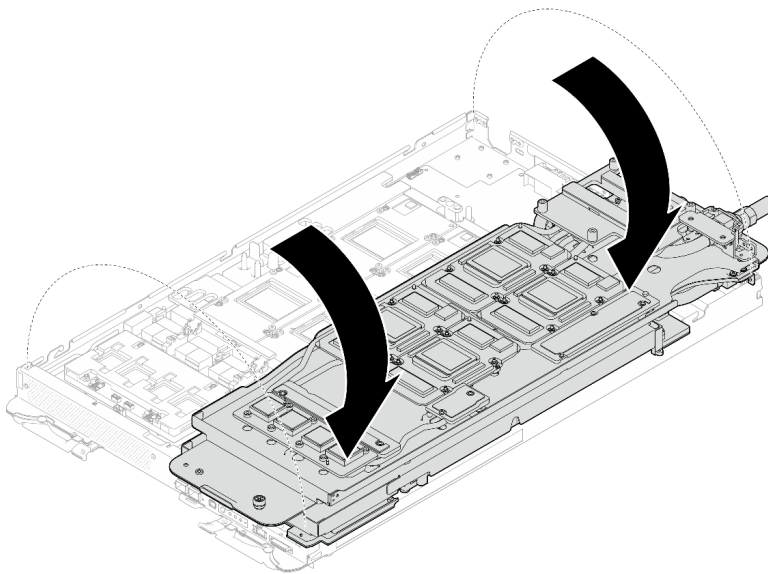
그림 393. GPU 노드 측 워터 루프를 컴퓨팅 노드 측 워터 루프 쪽으로 접기
