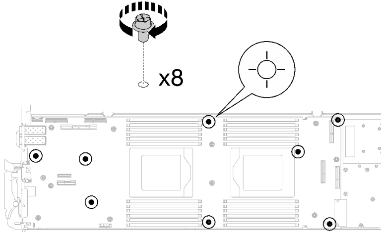
그림 307. 시스템 보드 나사 설치
