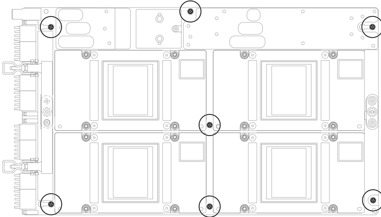
그림 375. GPU 보드 어셈블리에 M3 나사 설치
