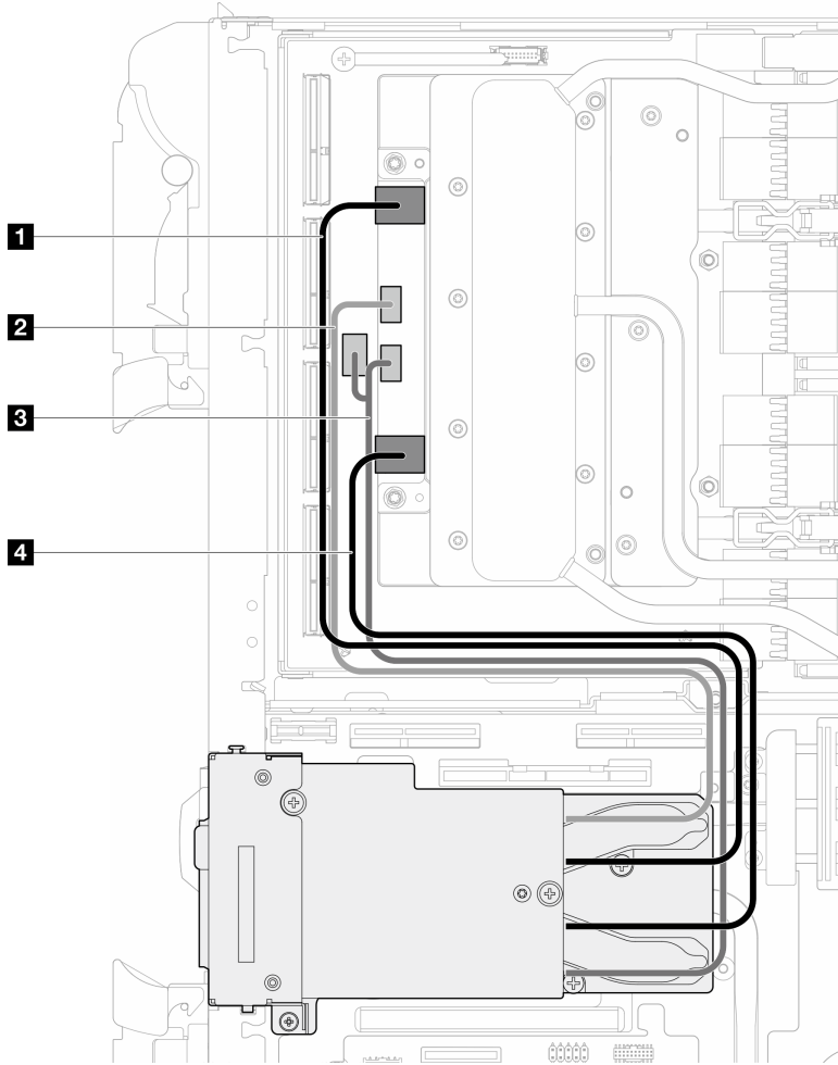
그림 414. OSFP 모듈 케이블을 네트워크 보드에서 연결 해제
