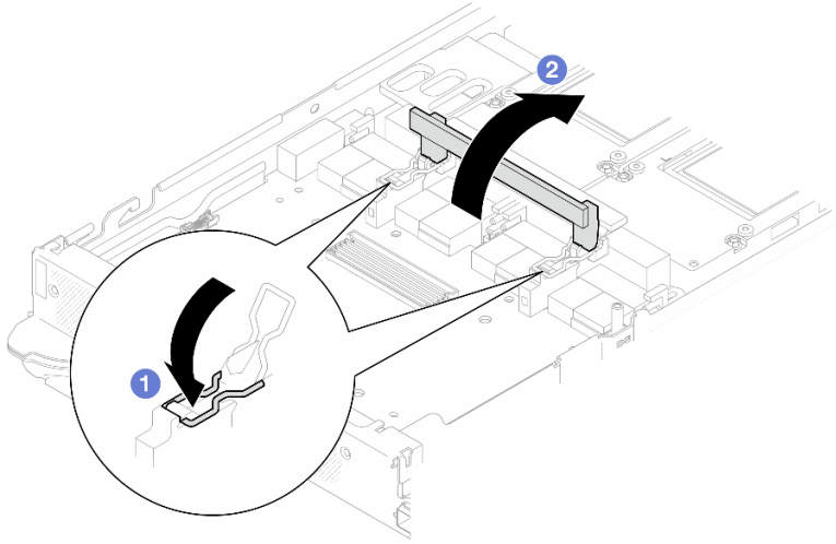
그림 317. 캐리어 보드를 GPU 보드에 고정
