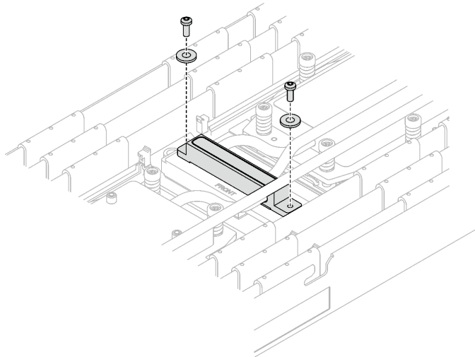
그림 185. 와셔가 있는 VR 냉각판 나사
