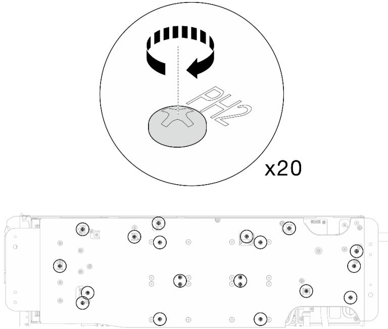
그림 22. 워터 루프 나사 및 빠른 연결 나사 제거(GPU 노드)
