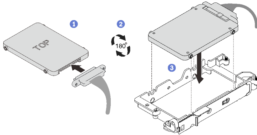
그림 98. 하단 드라이브 설치(7mm 드라이브)
