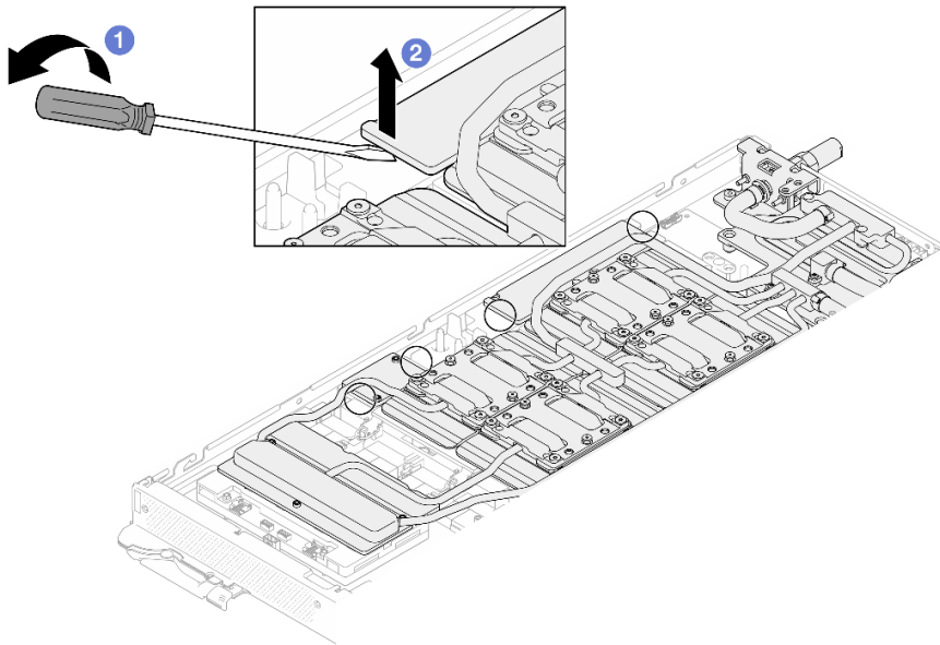
그림 328. 전면 및 후면 MISC 전도판을 GPU 보드에서 분리
