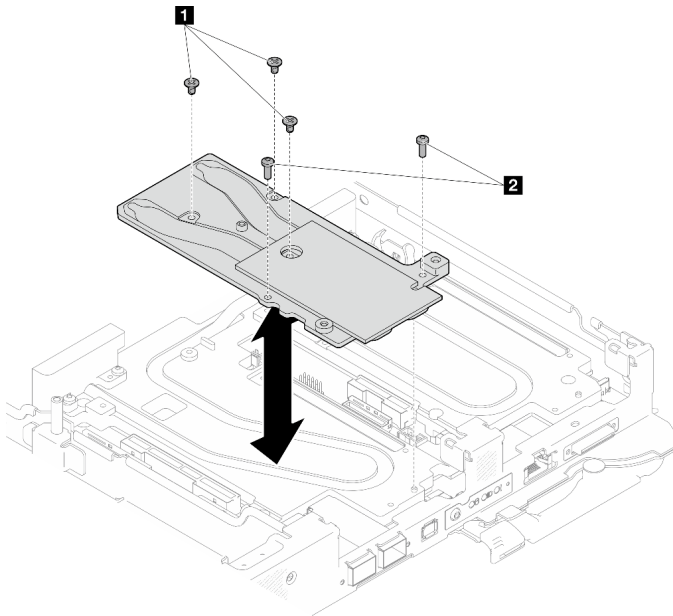
그림 208. OSFP 모듈 전도판 설치
