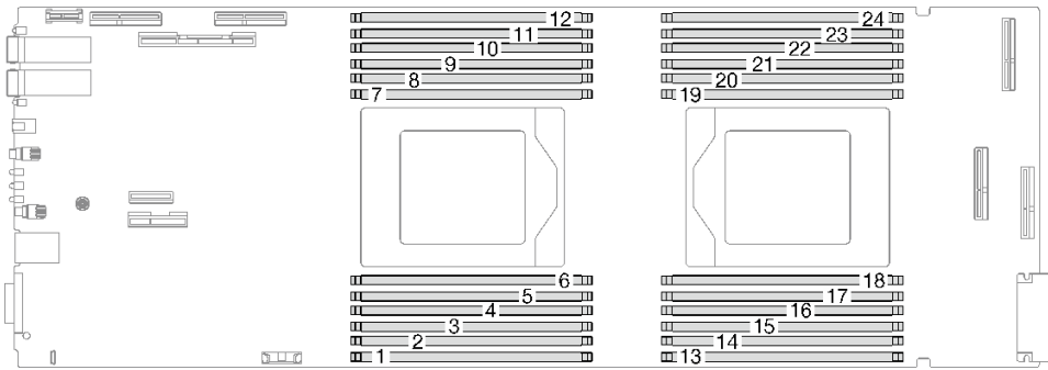
그림 159. 메모리 모듈 커넥터 위치
