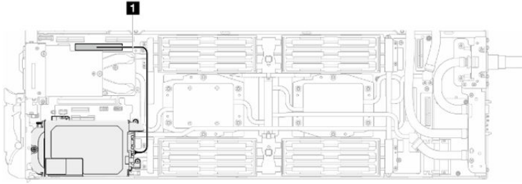
그림 121. E3.S 드라이브 케이블 연결 해제
