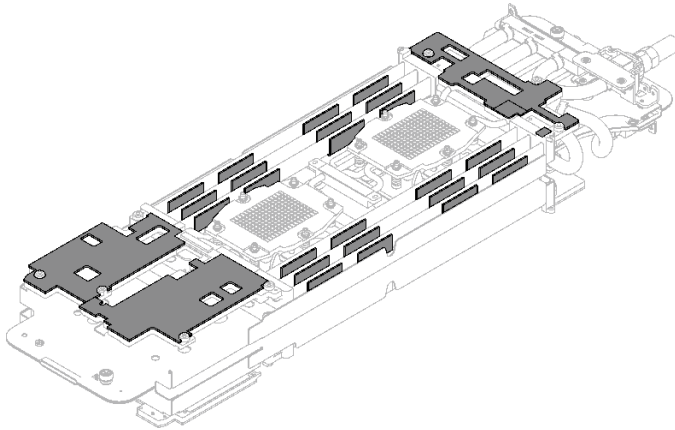
그림 227. 워터 루프 갭 패드(하단)
