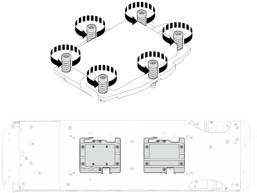
그림 247. 프로세서 냉각판 제거
