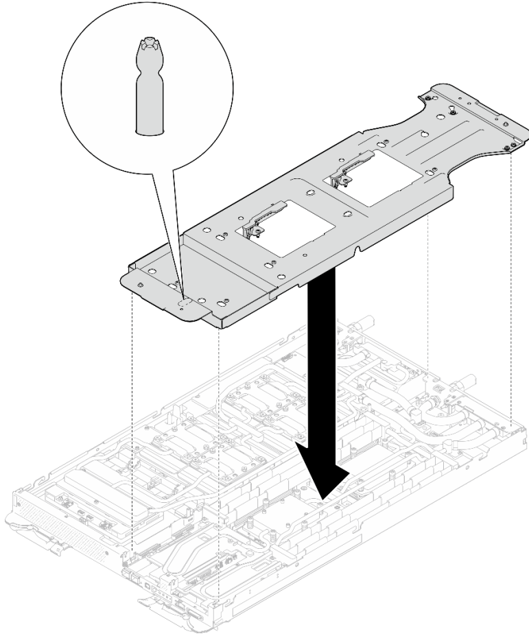
그림 189. 워터 루프 캐리어 설치(컴퓨팅 노드)
