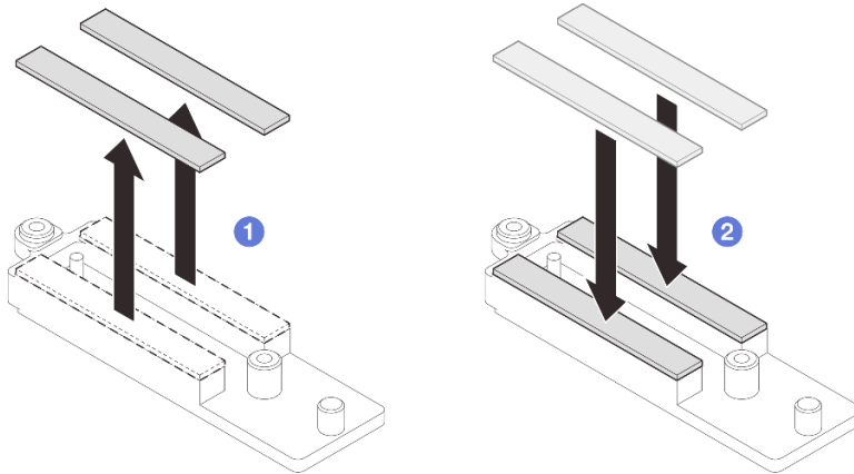
그림 305. VR 전도판 퍼티 패드 교체
