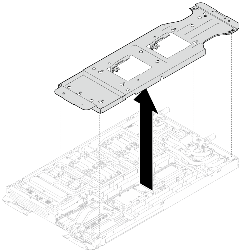
그림 233. 워터 루프 캐리어 제거(컴퓨팅 노드)
