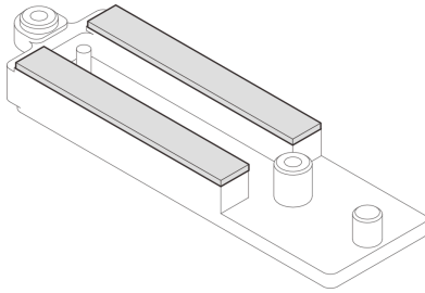
그림 70. VR 전도판 하단의 퍼티 패드
