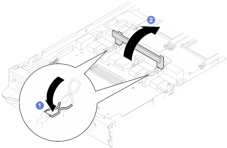
그림 365. 캐리어 보드를 GPU 보드에 고정
