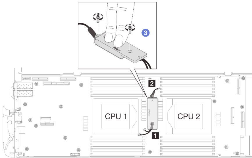
그림 299. 차폐 케이블 1/2 및 3 설치
