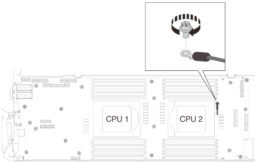
그림 284. 차폐 케이블 4 설치
