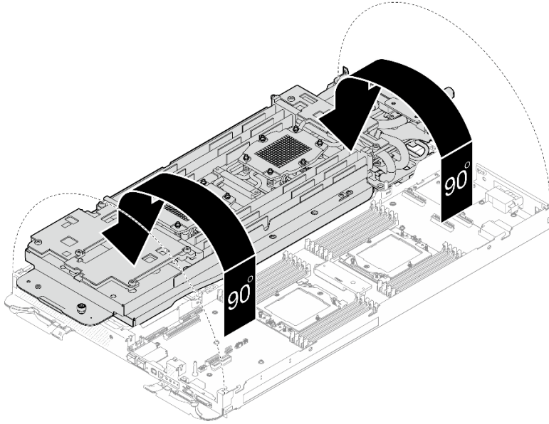
그림 251. 워터 루프 접기
