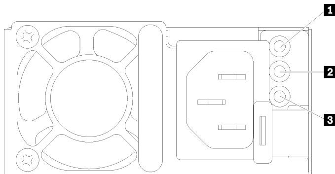
그림 459. AC 전원 공급 장치 LED
