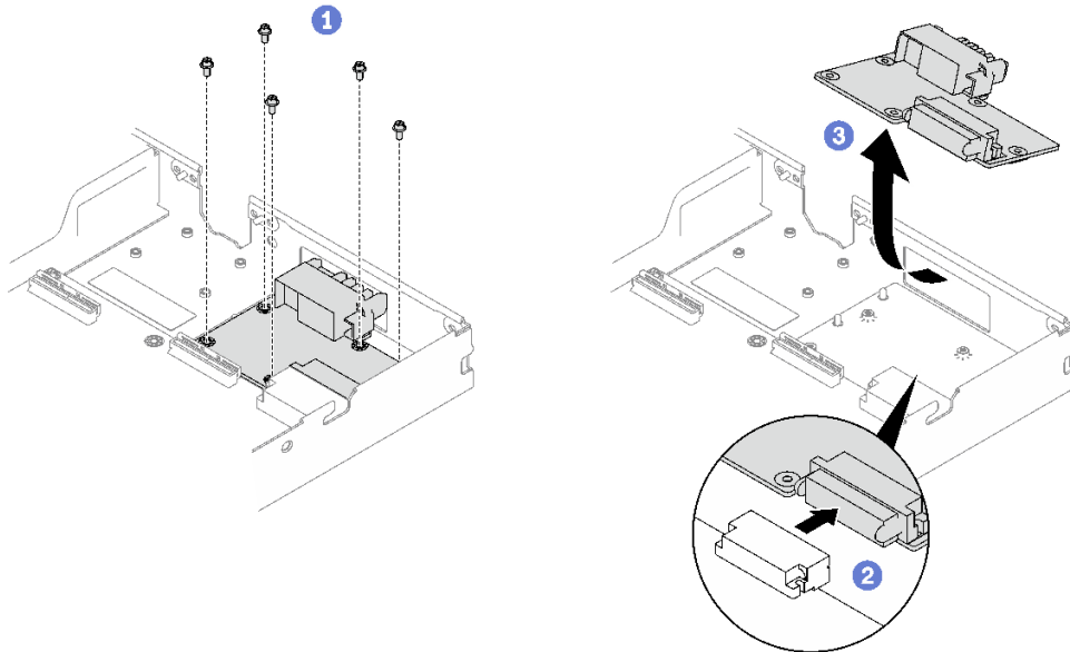
그림 193. 전원 분배 보드 제거
