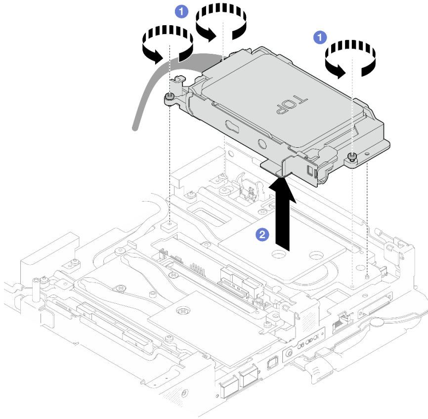
그림 89. 7mm 드라이브 케이지 어셈블리 2개 제거
