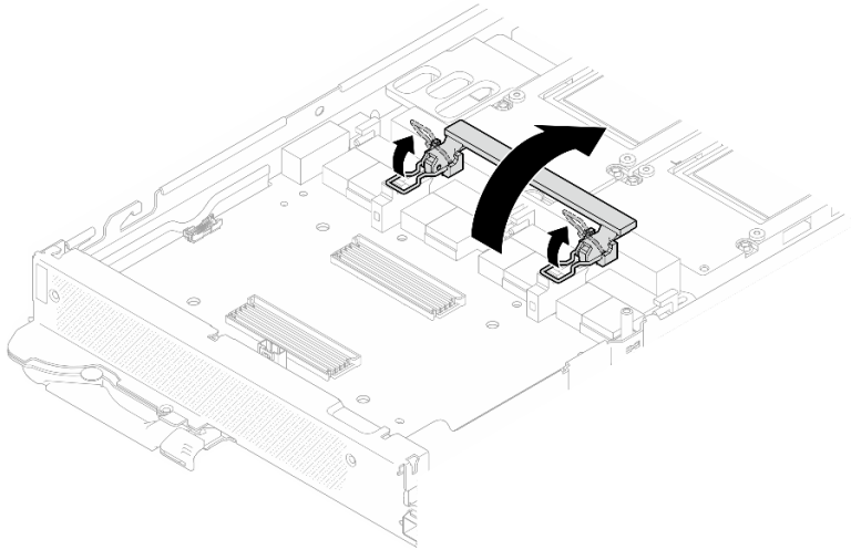
그림 315. GPU 보드 고정 클립 및 핸들 돌리기
