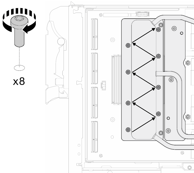
그림 63. 네트워크 카드 나사 설치
