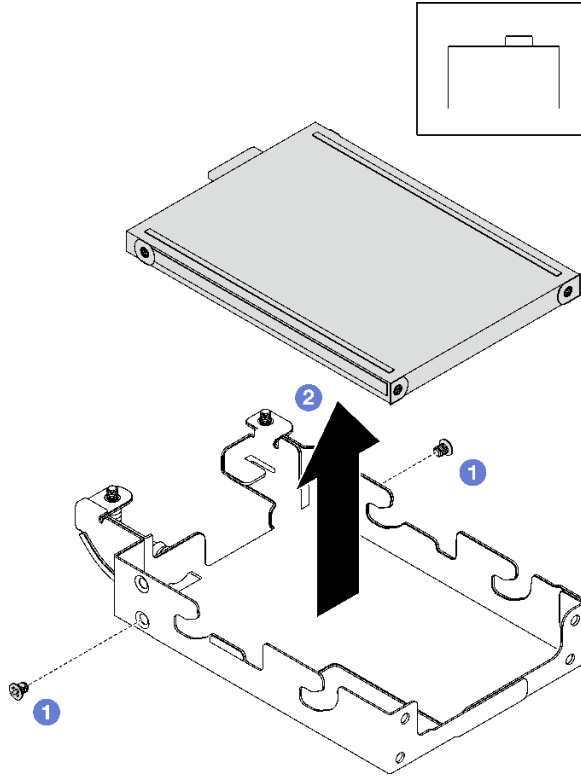
그림 129. 상단 E3.s 드라이브 제거
