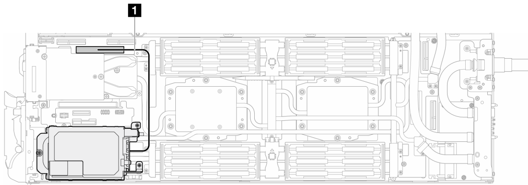
그림 141. E3.S 드라이브 케이블 배선
