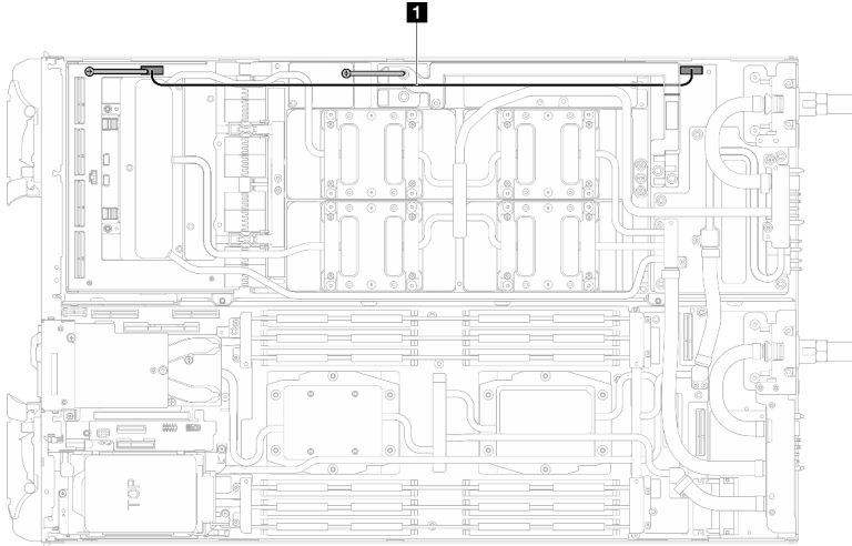
그림 415. 캐리어 보드 전원 케이블 제거
