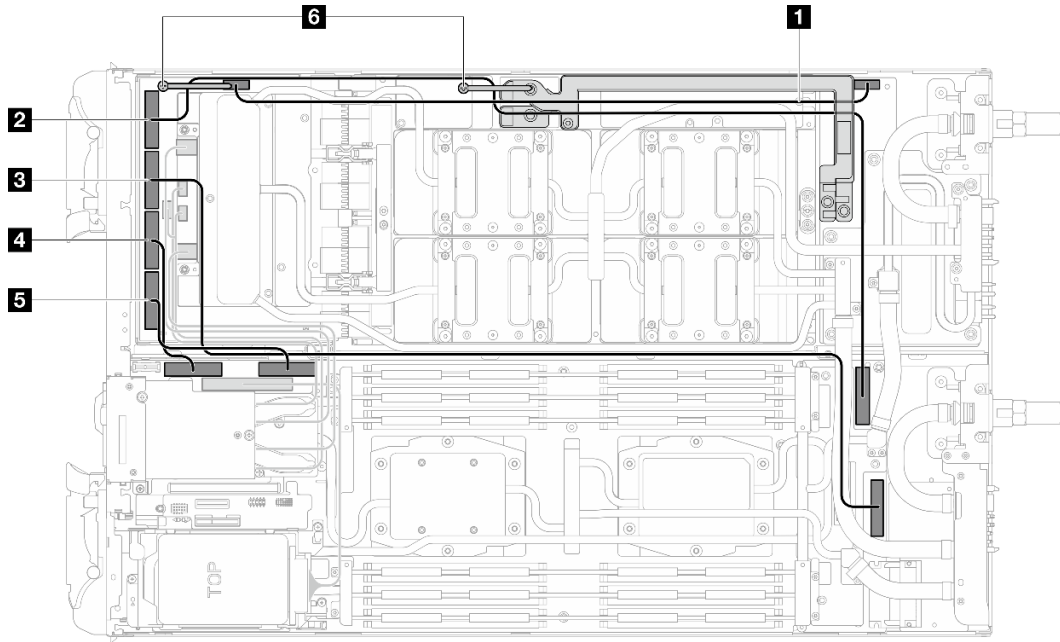
그림 453. 프로세서 2개 구성 케이블 배선
