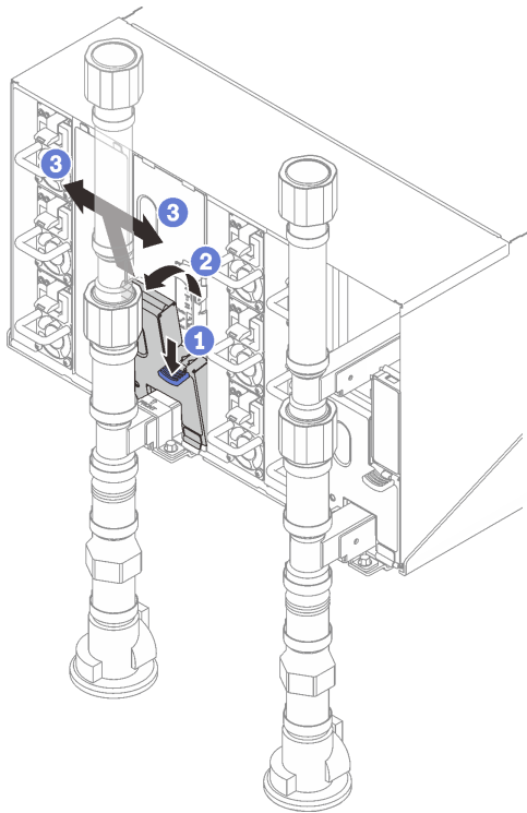
그림 465. 하단 EMC 실드 제거
