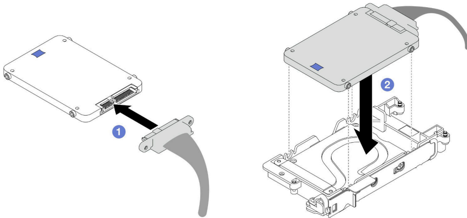
그림 114. 아래쪽 드라이브 설치
