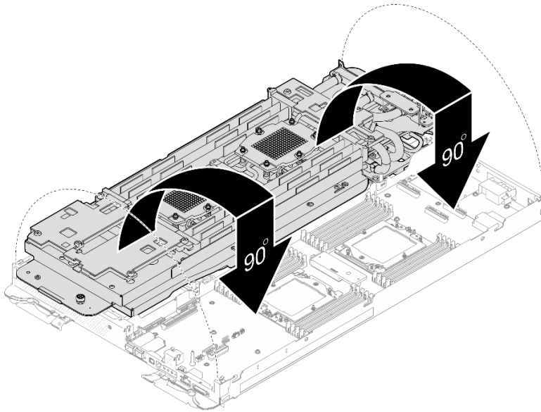
그림 231. 워터 루프 설치
