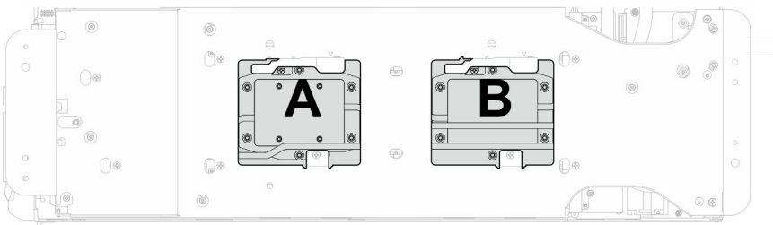
그림 53. 프로세서 냉각판 설치
