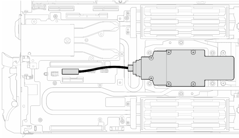
그림 142. M.2 백플레인 어셈블리 케이블 제거
