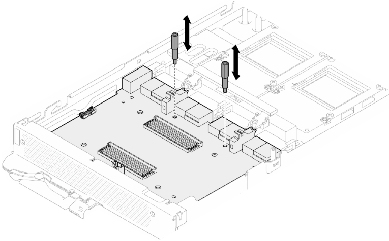
그림 367. 캐리어 보드 스탠드오프 제거
