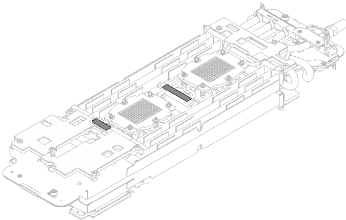
그림 229. 워터 루프 퍼티 패드
