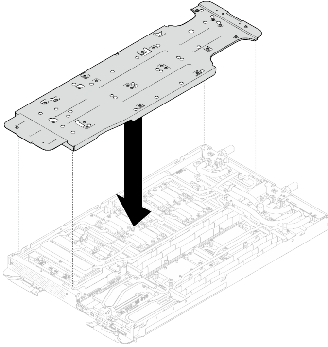
그림 331. 워터 루프 캐리어 설치(GPU 노드)
