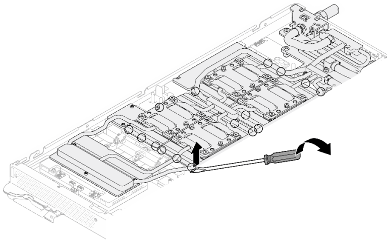
그림 330. GPU에서 GPU 냉각판 분리
