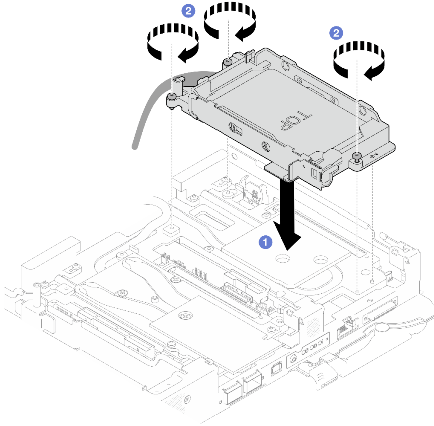
그림 104. 7mm 드라이브 케이지 어셈블리 1개 설치
