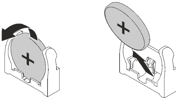
그림 80. CMOS 배터리 제거
