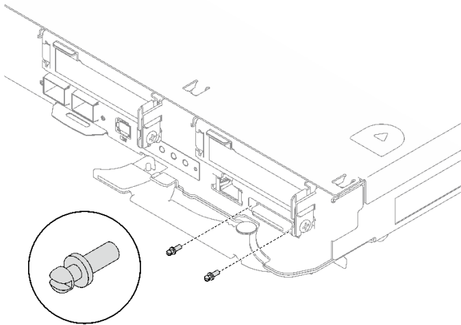
그림 308. KVM 나사 설치
