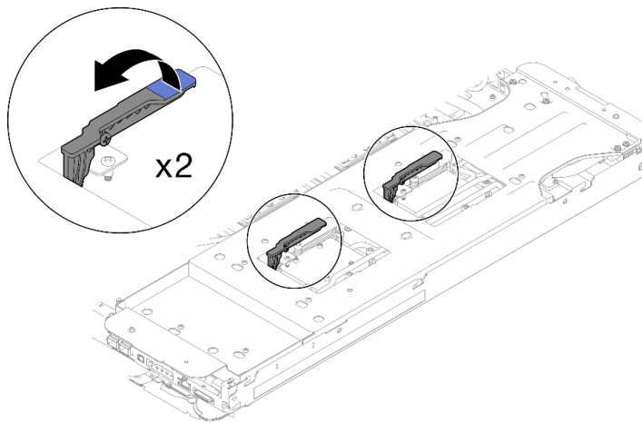
그림 36. 프로세서에서 워터 루프 분리
