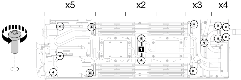
그림 31. 워터 루프 나사 제거
