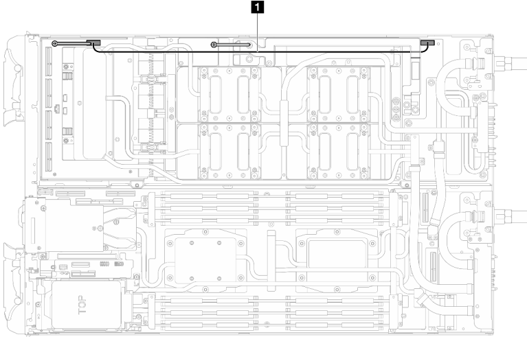
그림 321. 캐리어 보드 전원 케이블 제거
