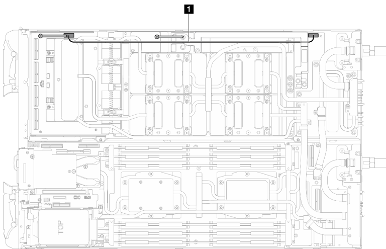
그림 11. 캐리어 보드 전원 케이블 제거
