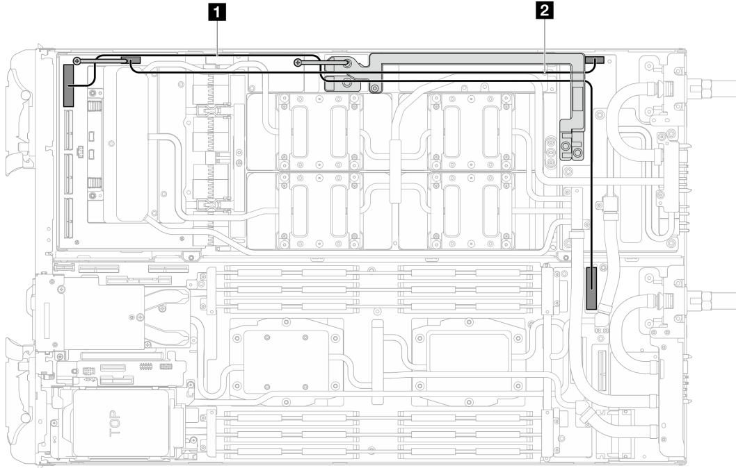
그림 310. 캐리어 보드 전원 케이블 및 MCIO 1 케이블 배선
