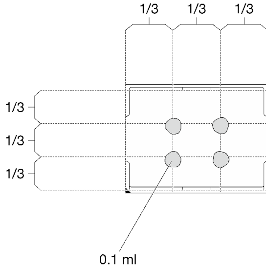
그림 195. 열전도 그리스 도포
