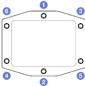
그림 32. 프로세서 냉각판 레이블
