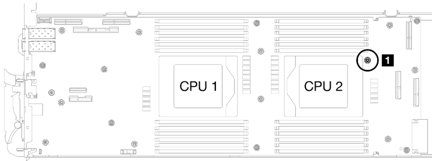
그림 300. 차폐 케이블 4의 나사 구멍 위치
