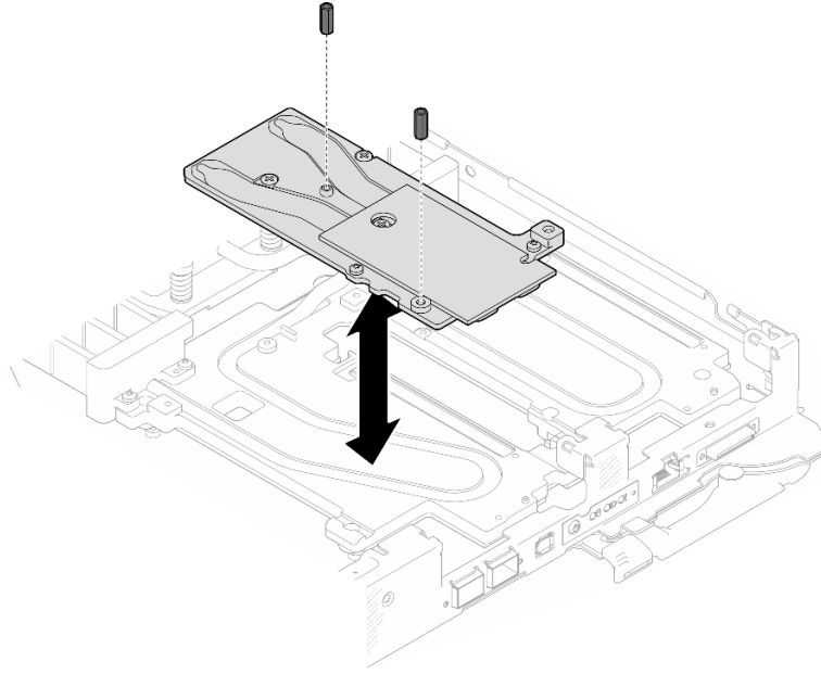
그림 209. OSFP 모듈 전도판 육각 나사 설치
