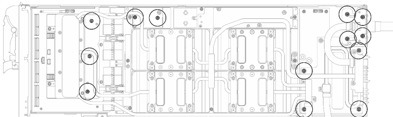
그림 410. 워터 루프 Torx T10 나사 설치(GPU 노드)
