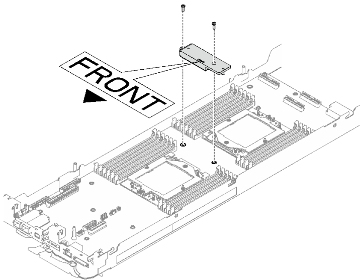
그림 78. VR 전도판 제거
