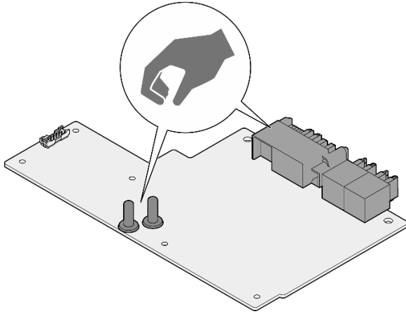
그림 398. SD665-N V3 GPU 전원 분배 보드 터치 포인트
