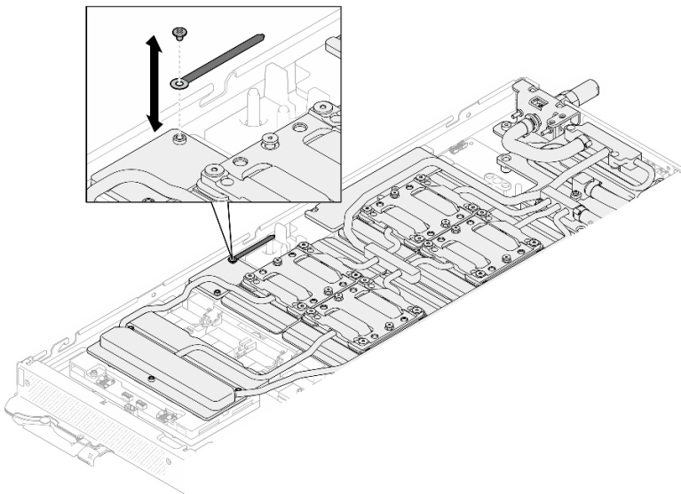
그림 322. 케이블 타이 제거
