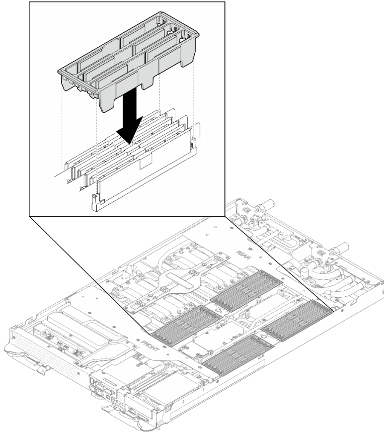
그림 164. DIMM 덮개 설치
