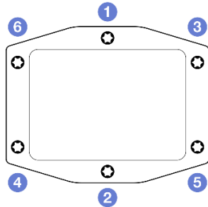
그림 216. 프로세서 냉각판 레이블
