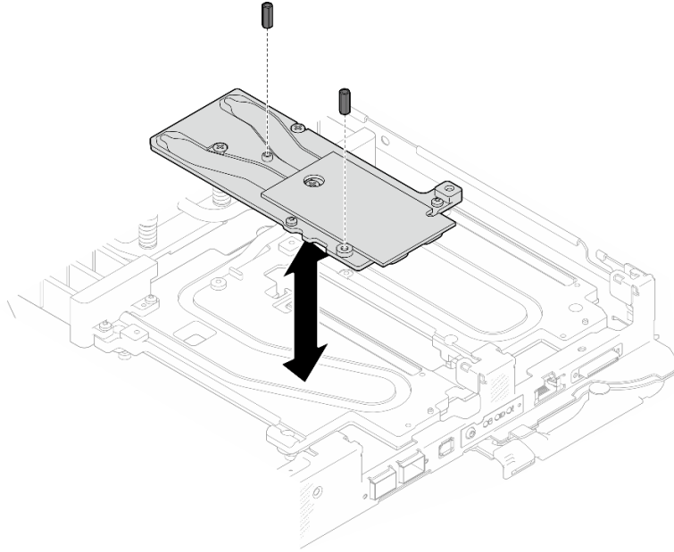
그림 211. OSFP 모듈 전도판 육각 나사 제거
