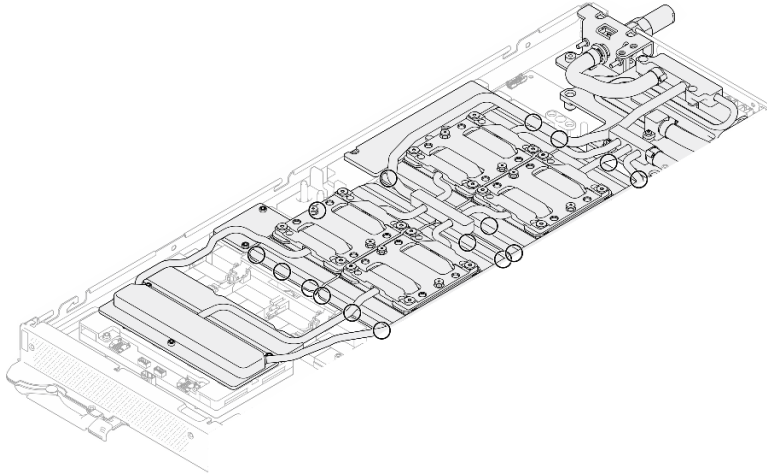
그림 329. GPU 냉각판 분리를 위한 노치
