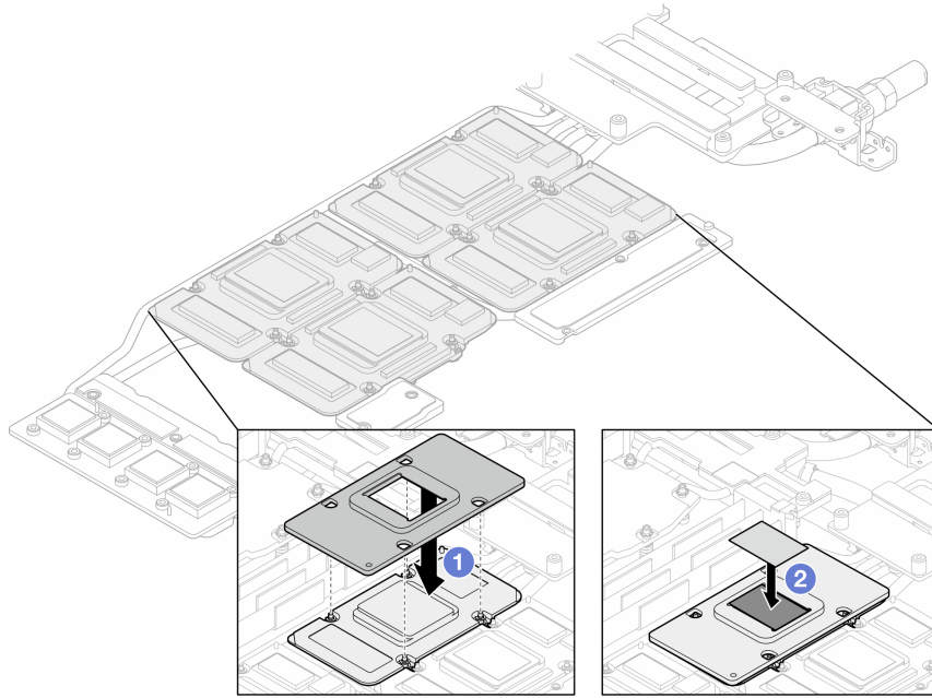
그림 434. 워터 루프 GPU 냉각판 PCM 교체(GPU 노드)
