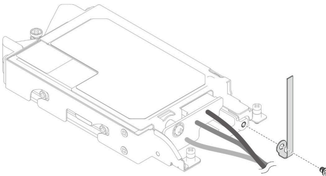
그림 125. 케이블 타이 제거
