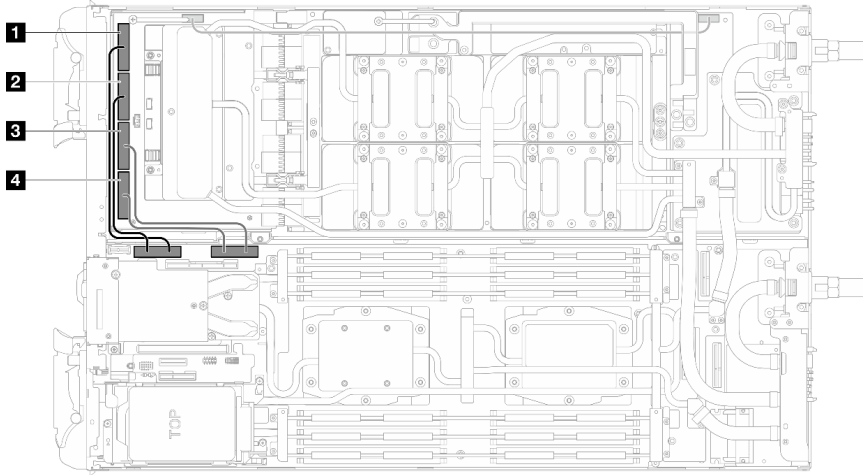
그림 178. 프로세서 1개 구성 - 모든 MCIO 케이블을 캐리어 보드에 연결
