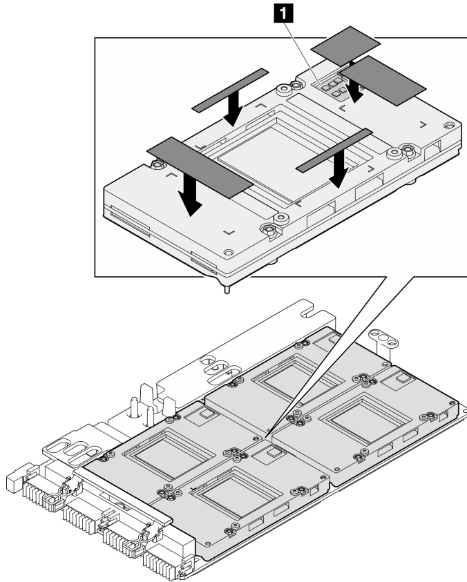
그림 403. GPU 퍼티 패드 교체
