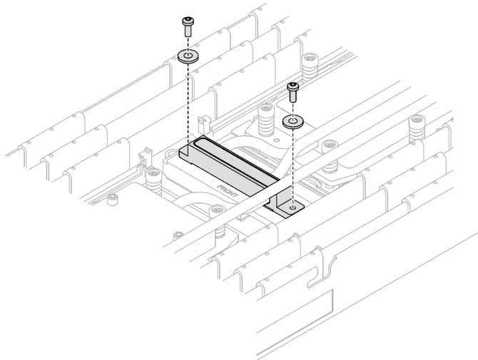
그림 30. 와셔가 있는 VR 냉각판 나사
