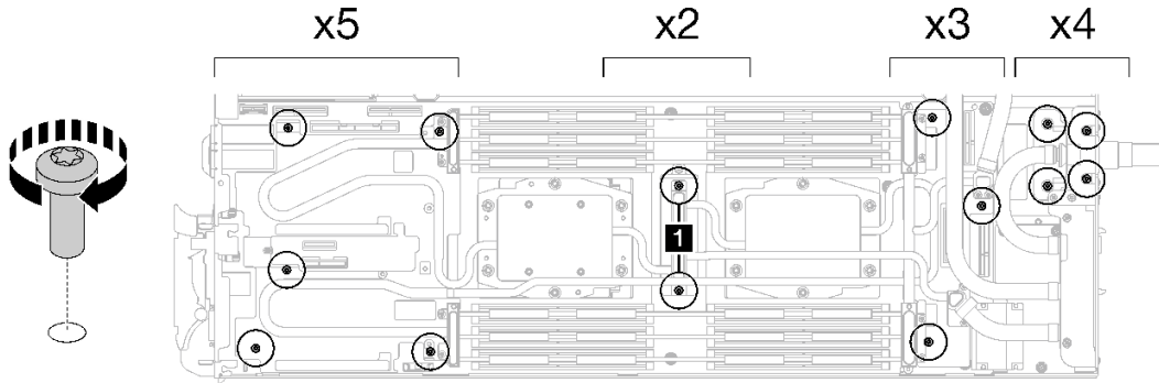
그림 205. 워터 루프 나사 및 퀵 커넥트 나사 설치
