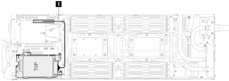
그림 166. 드라이브 케이블 연결 해제
