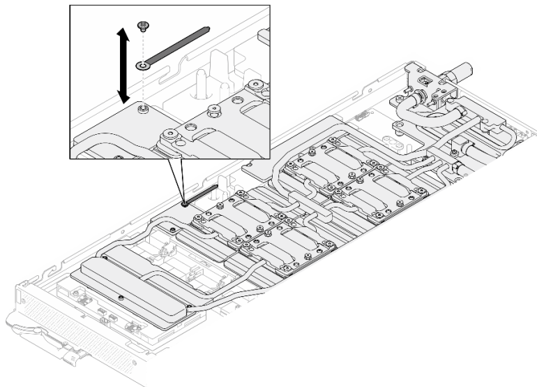
그림 412. 케이블 타이 설치
