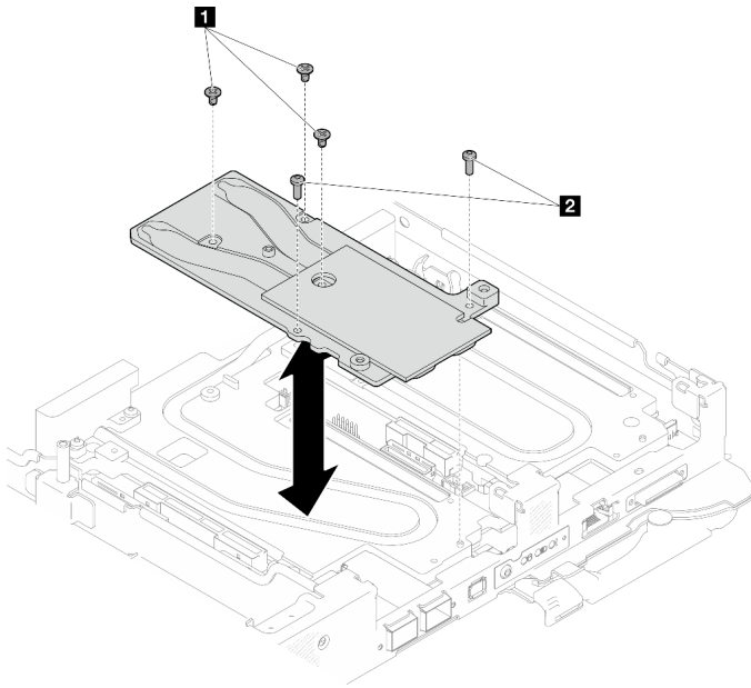
그림 268. OSFP 모듈 전도판 설치
