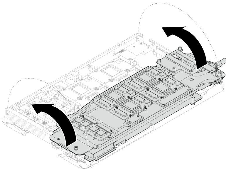
그림 404. 워터 루프를 GPU 노드에 펼치기
