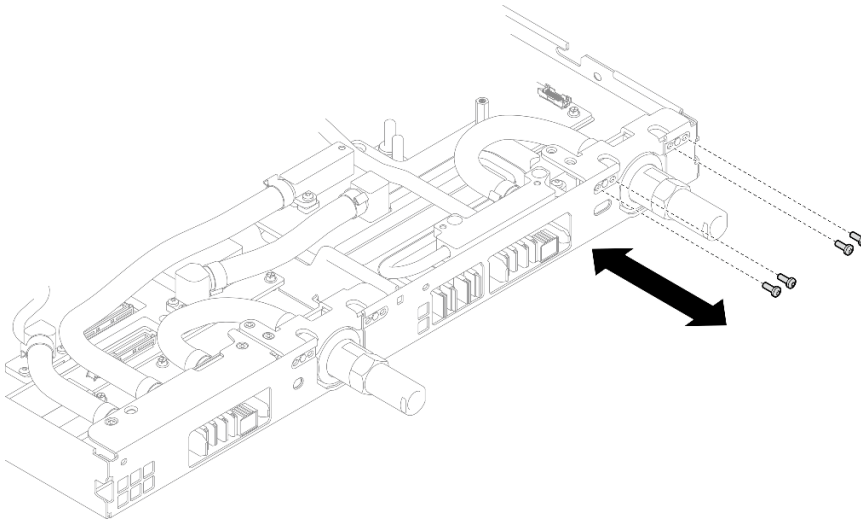
그림 385. 퀵 커넥트 나사 제거(GPU 노트)
