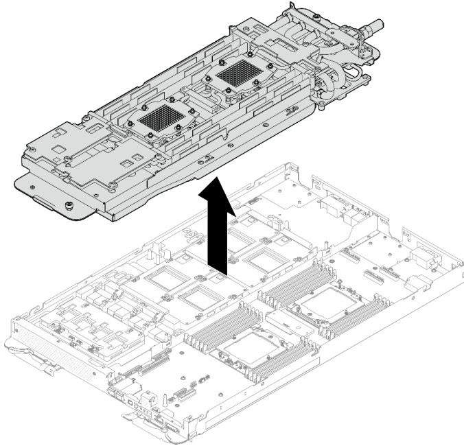
그림 39. 워터 루프 제거
