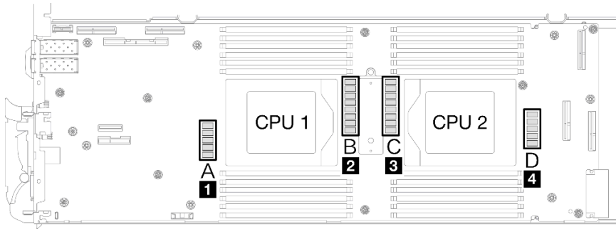
그림 288. 시스템 보드의 인덕터 위치
