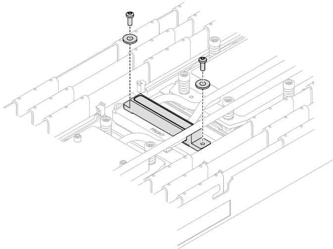
그림 244. 와셔가 있는 VR 냉각판 나사
