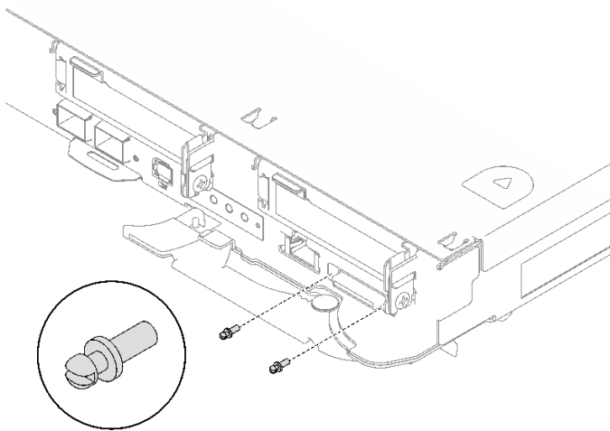
그림 270. KVM 나사 제거
