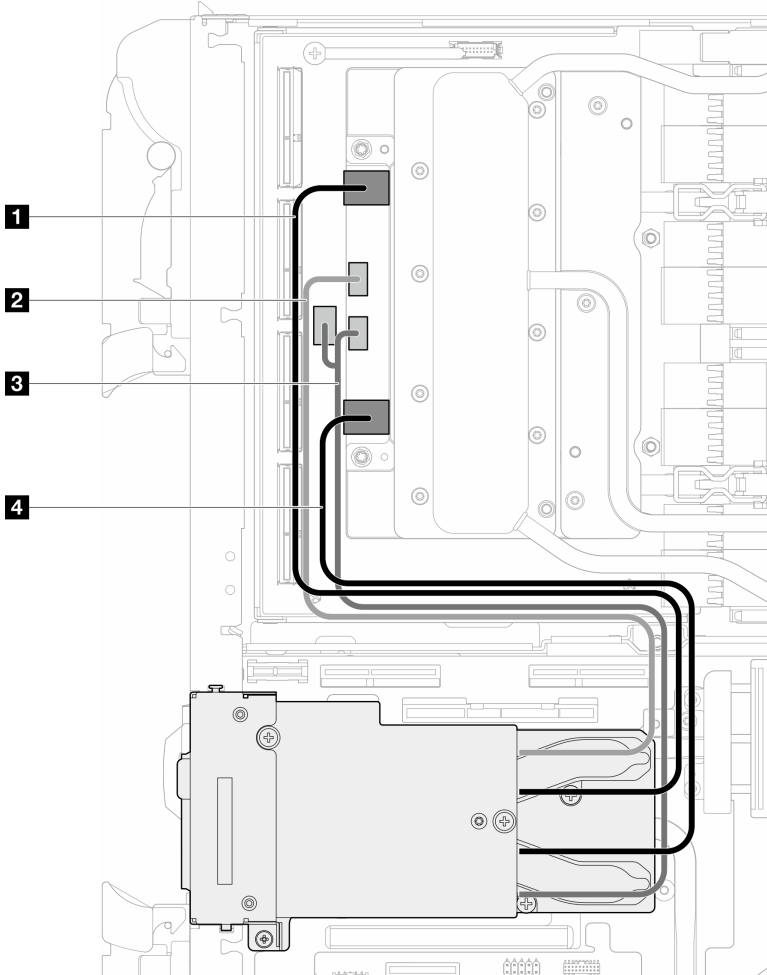
그림 170. OSFP 모듈 케이블을 네트워크 보드에서 연결 해제
