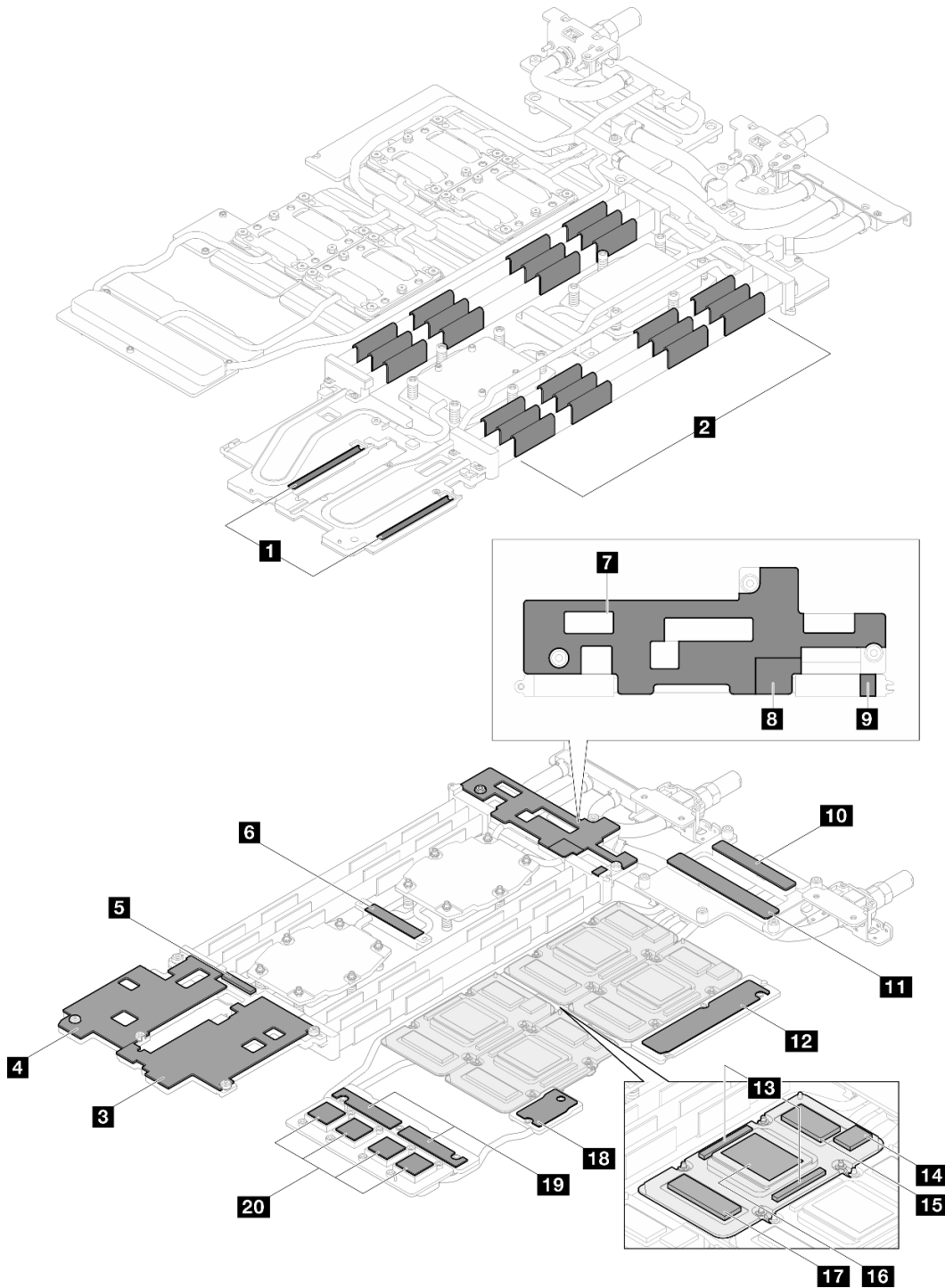
그림 2. 워터 루프 및 GPU 노드 - 갭 패드/퍼티 패드 식별 및 위치
