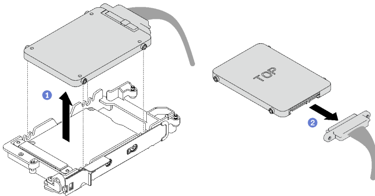
그림 91. 7mm 드라이브 1개 제거
