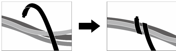
그림 451. 케이블 타이 묶기
