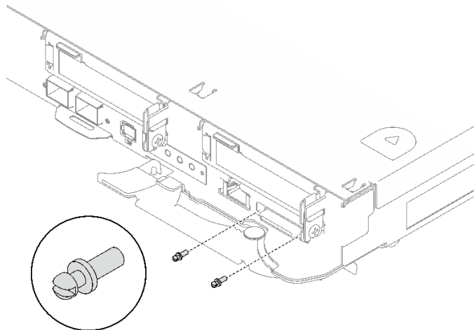
그림 304. KVM 나사 설치
