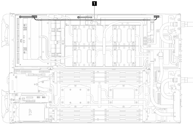
그림 381. 캐리어 보드 전원 케이블 제거
