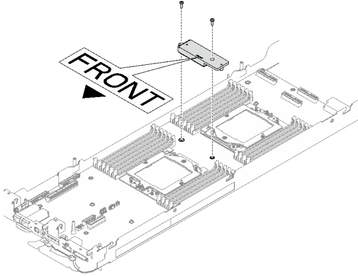
그림 69. VR 전도판 제거
