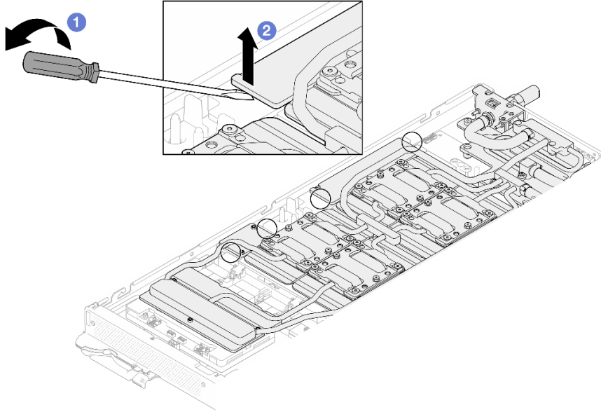
그림 388. 전면 및 후면 MISC 전도판을 GPU 보드에서 분리
