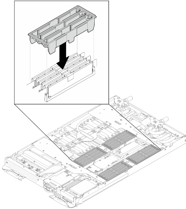
그림 157. DIMM 덮개 설치
