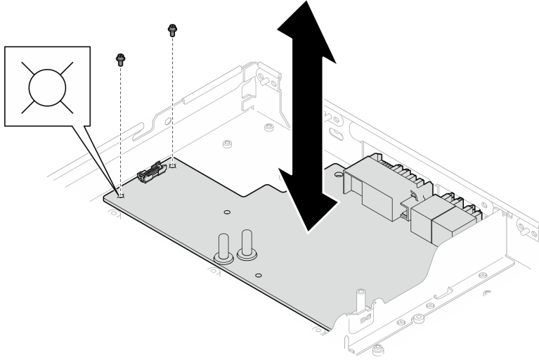
그림 396. GPU 전원 분배 보드 나사 제거
