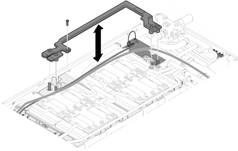
그림 309. 버스 바 제거
