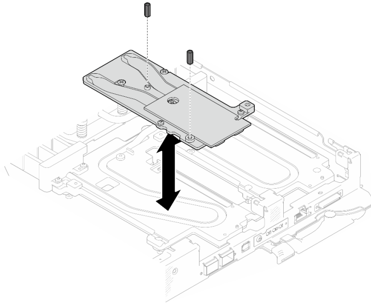
그림 59. OSFP 모듈 전도판 육각 나사 설치
