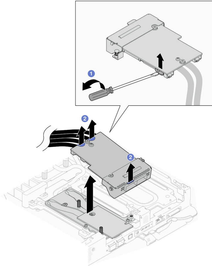
그림 172. OSFP 모듈 제거
