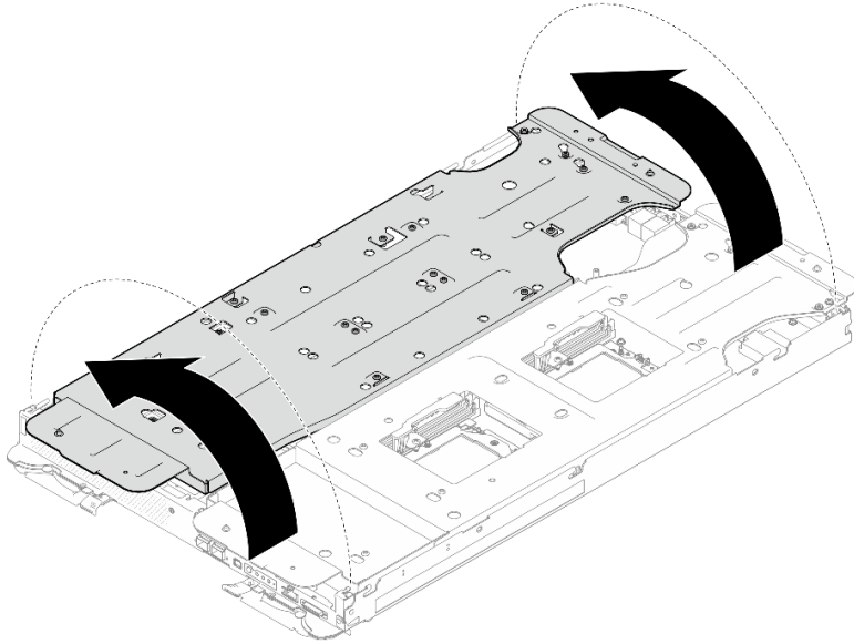
그림 50. 워터 루프 펼치기
