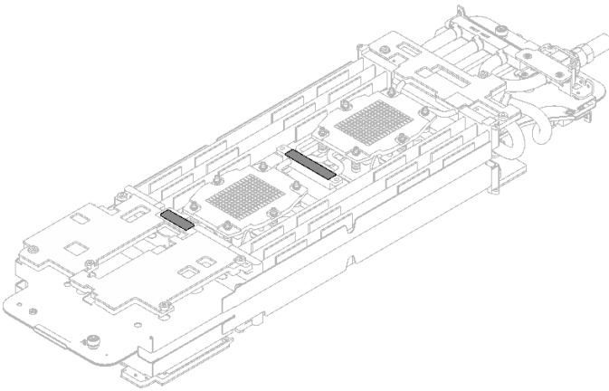
그림 258. 워터 루프 퍼티 패드
