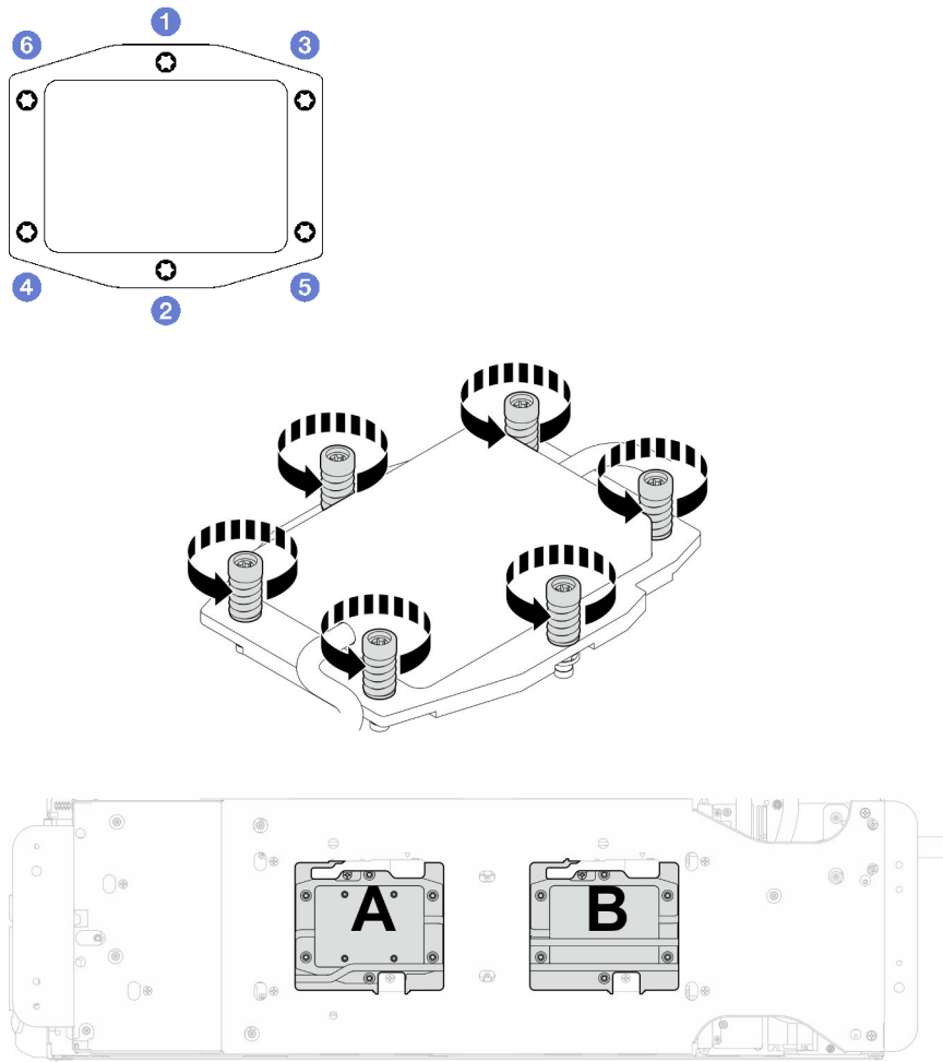
그림 203. 프로세서 냉각판 설치
