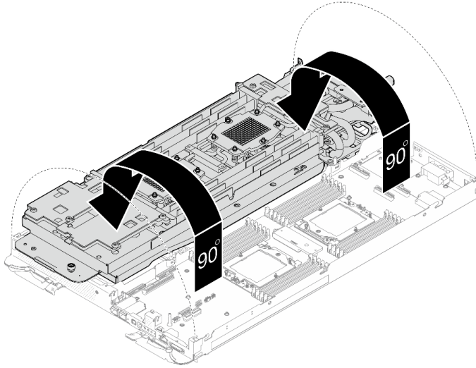
그림 37. 워터 루프 접기
