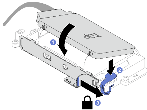
그림 99. 상단 드라이브 설치(7mm 드라이브)
