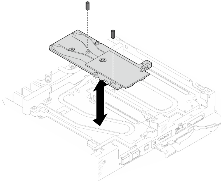
그림 27. OSFP 모듈 전도판 육각 나사 제거
