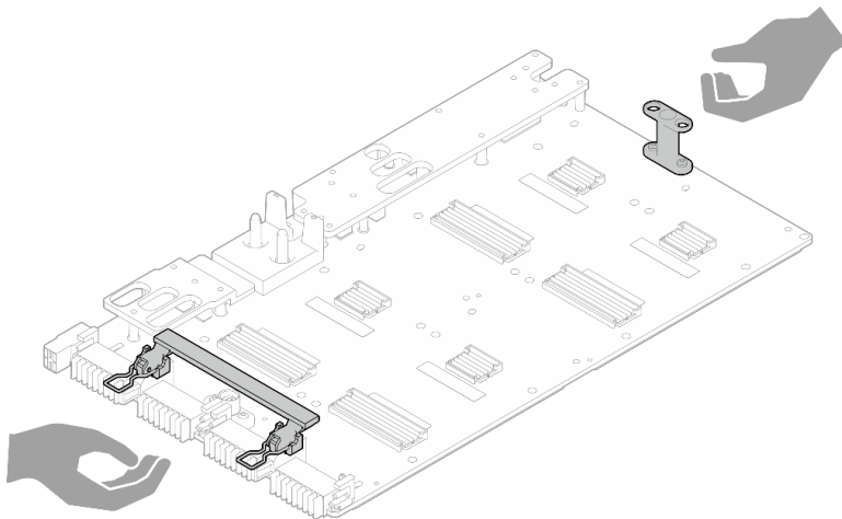
그림 360. 패키지 상자에서 GPU 보드 제거
