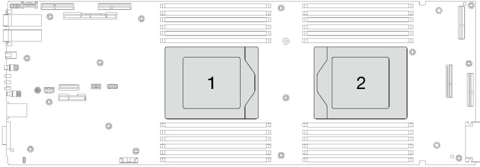
그림 223. 프로세서 위치
