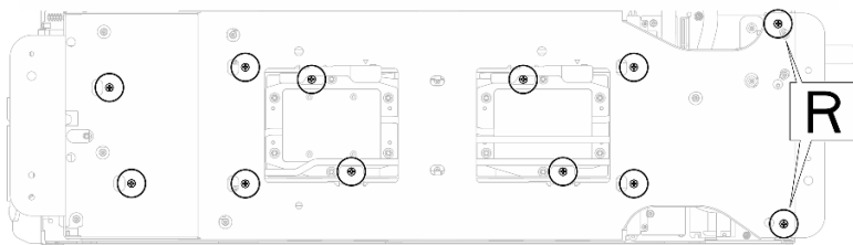
그림 51. 워터 루프 캐리어 나사 풀기
