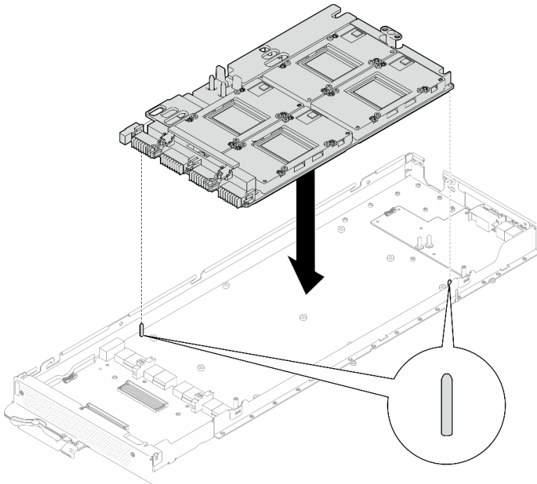
그림 374. 노드에 GPU 보드 어셈블리 설치
