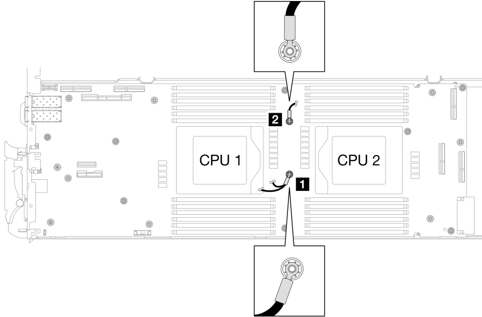
그림 279. 차폐 케이블 1/2 및 차폐 케이블 3을 나사 구멍에 맞추기
