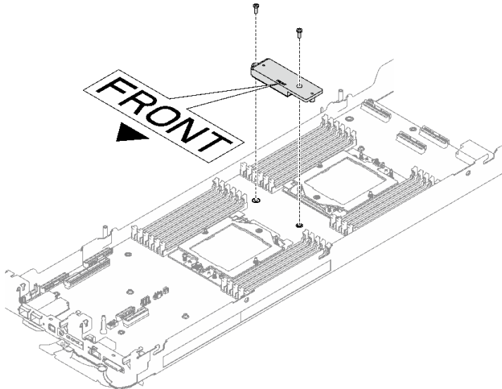
그림 76. VR 전도판 제거
