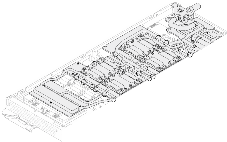
그림 389. GPU 냉각판 분리를 위한 노치
