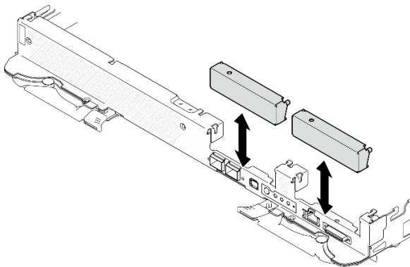
그림 100. 빈 베젤 필터 설치
