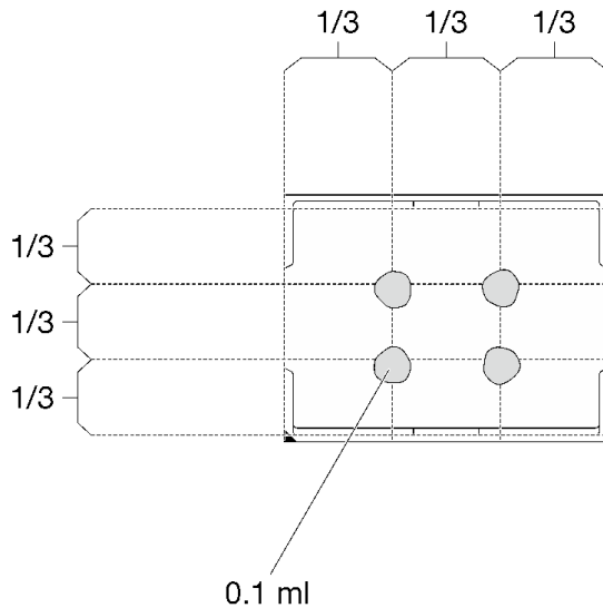
그림 225. 열전도 그리스 도포
