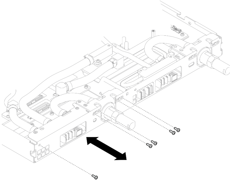
그림 206. 퀵 커넥트 나사 설치(컴퓨팅 노드)
