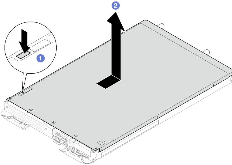
그림 5. 트레이 덮개 제거
