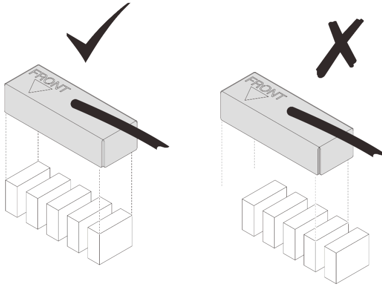
그림 291. 차폐 케이스로 인덱터 덮기
