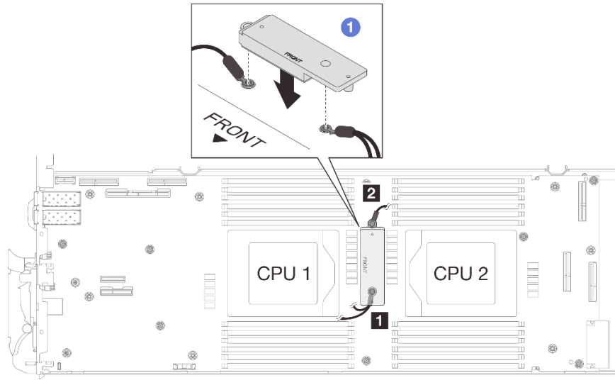
그림 73. VR 전도판, 차폐 케이블 및 시스템 보드 나사 구멍 맞추기
