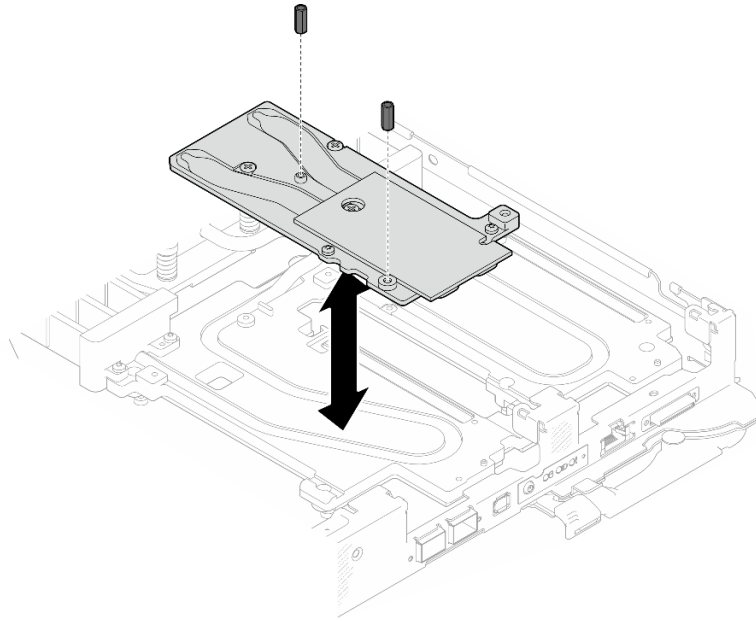
그림 182. OSFP 모듈 전도판 육각 나사 제거
