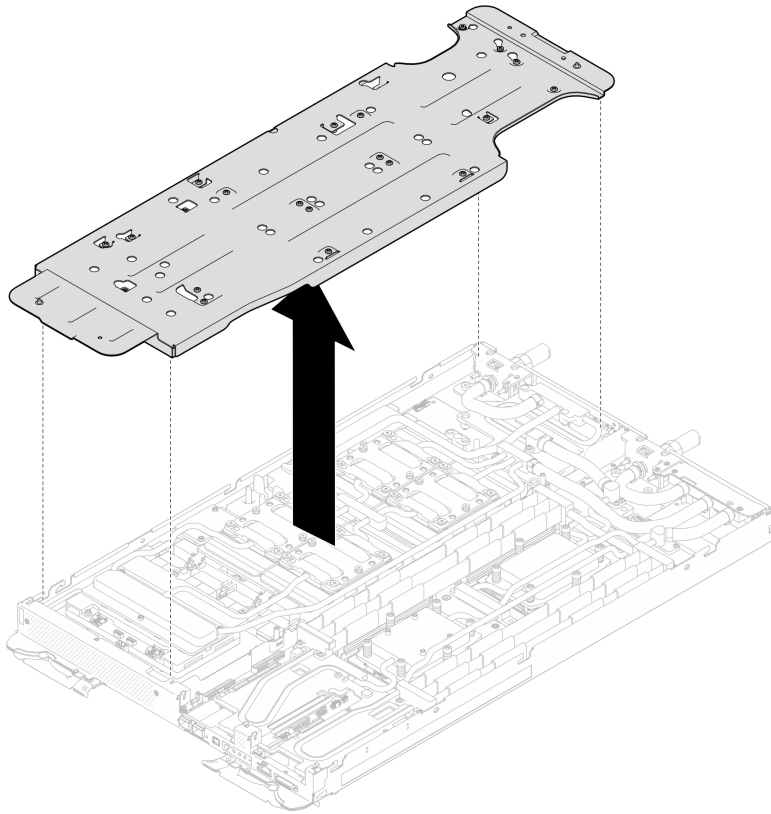
그림 439. 워터 루프 캐리어 제거(GPU 노드)
