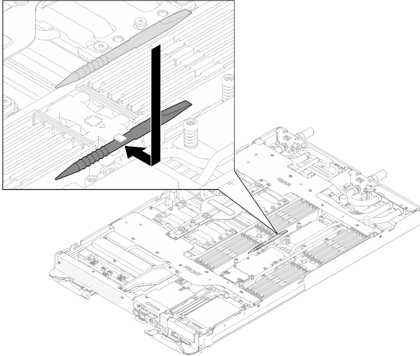
그림 165. 메모리 모듈 도구
