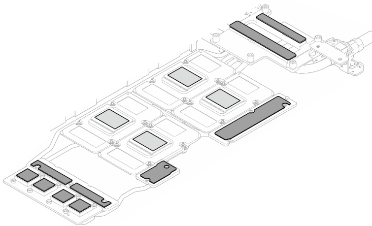
그림 341. 워터 루프 퍼티 패드 교체(GPU 노드)
