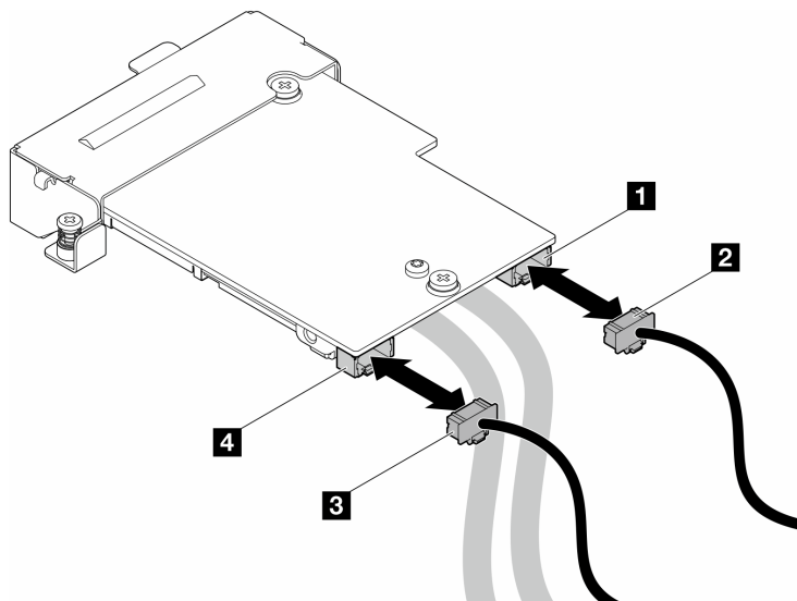
그림 175. OSFP 모듈 전원 케이블 설치
