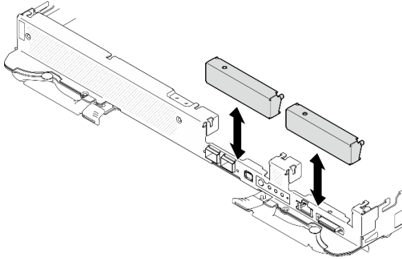
그림 116. 빈 베젤 필러 설치
