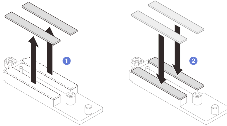
그림 275. VR 전도판 페리 패드 교체
