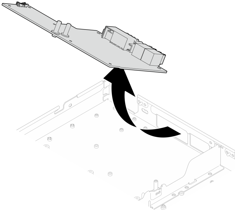
그림 397. GPU 전원 분배 보드 제거
