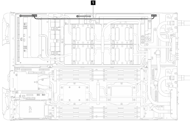
그림 413. 캐리어 보드 전원 케이블 연결
