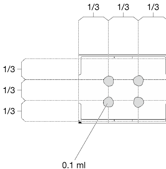
그림 254. 열전도 그리스 도포
