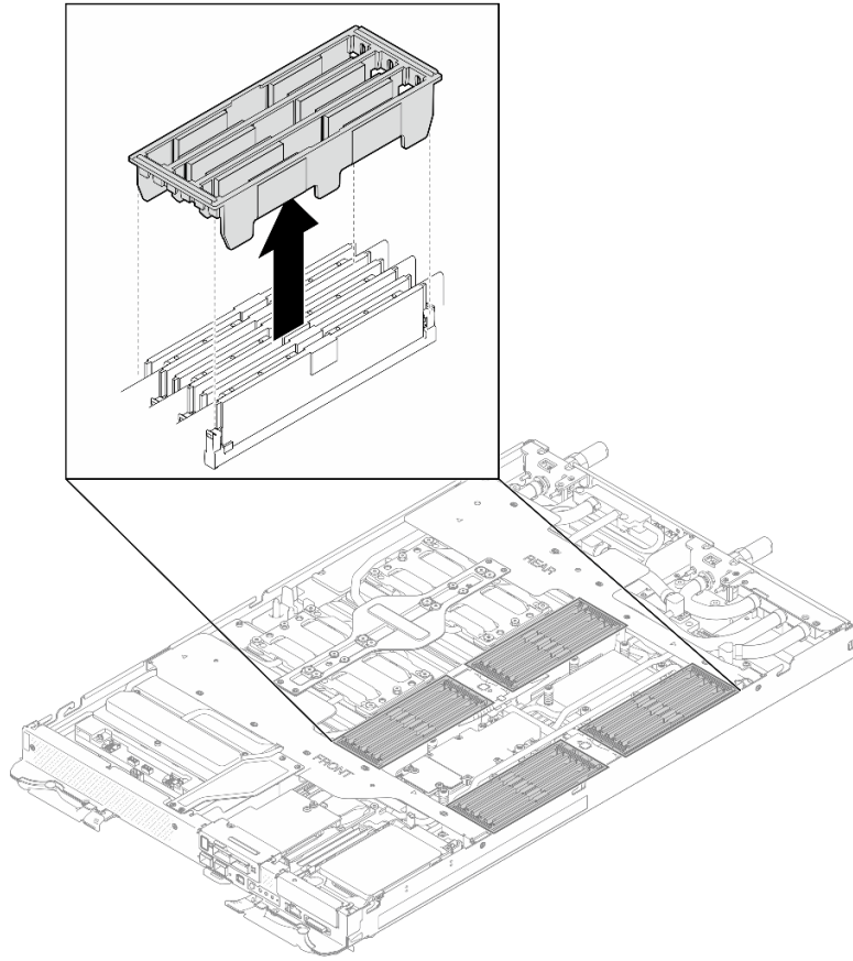
그림 161. DIMM 덮개 제거
