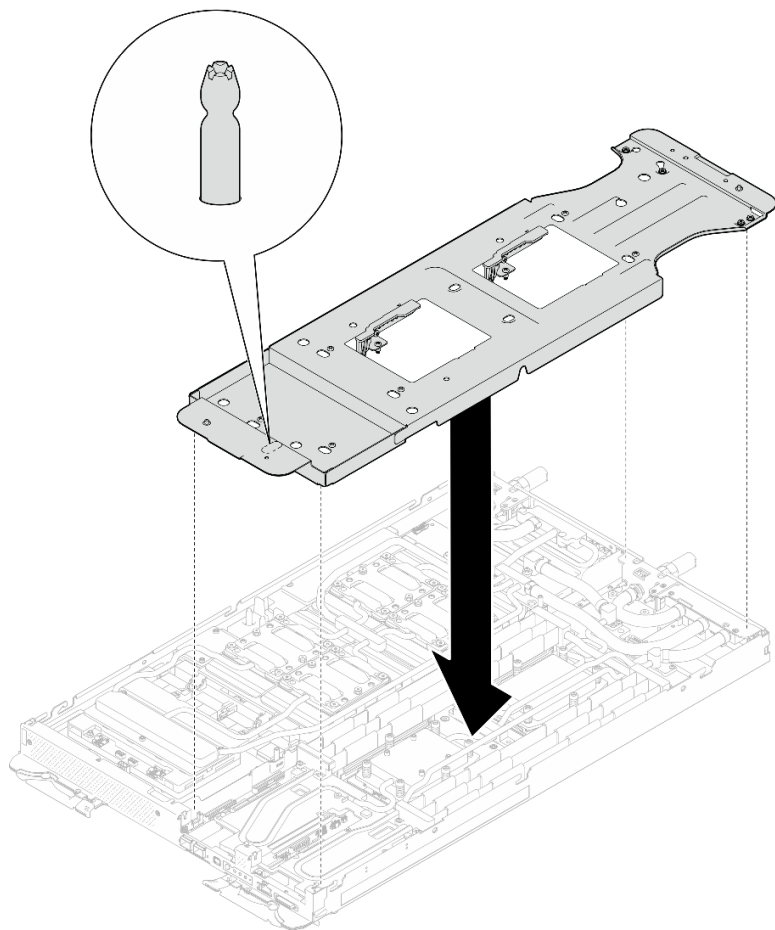
그림 34. 워터 루프 캐리어 설치(컴퓨팅 노드)
