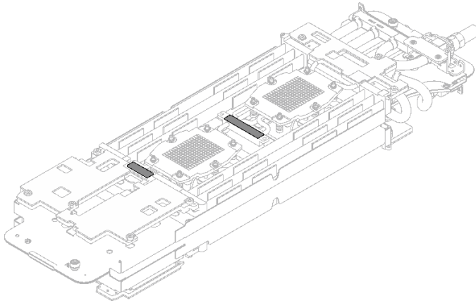
그림 198. 워터 루프 퍼티 패드
