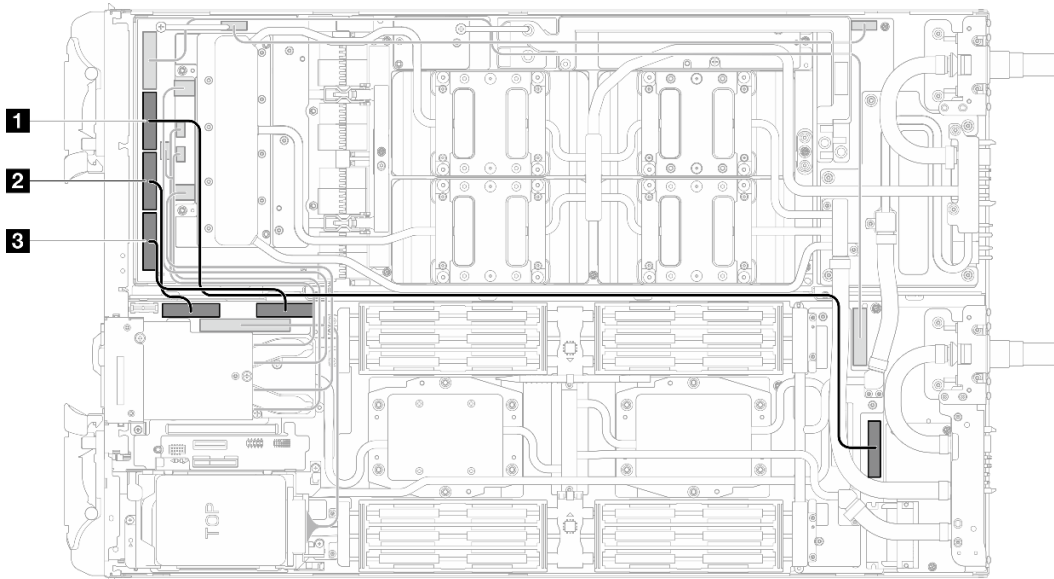
그림 169. 프로세서 2개 구성 - MCIO 2, MCIO 3 및 MCIO 4 케이블을 연결 해제
