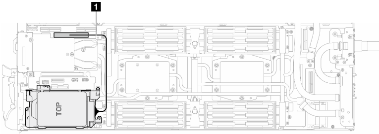
그림 180. 드라이브 케이블 연결
