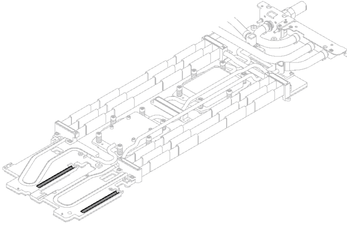
그림 228. 워터 루프 갭 패드(상단)
