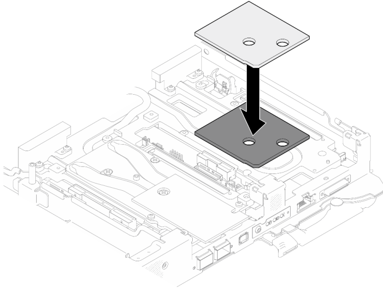
그림 118. 갭 패드 교체
