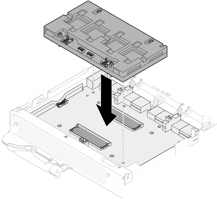
그림 432. 네트워크 보드 설치
