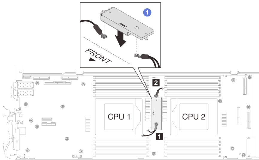
그림 280. VR 전도판, 차폐 케이블 및 시스템 보드 나사 구멍 맞추기
