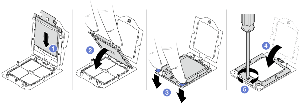
그림 224. 프로세서 설치
