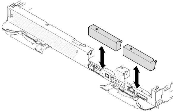
그림 138. 빈 베젤 필러 설치
