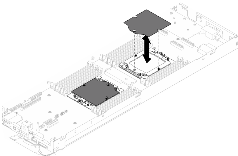
그림 252. 프로세서 소켓 보호 필름 제거
