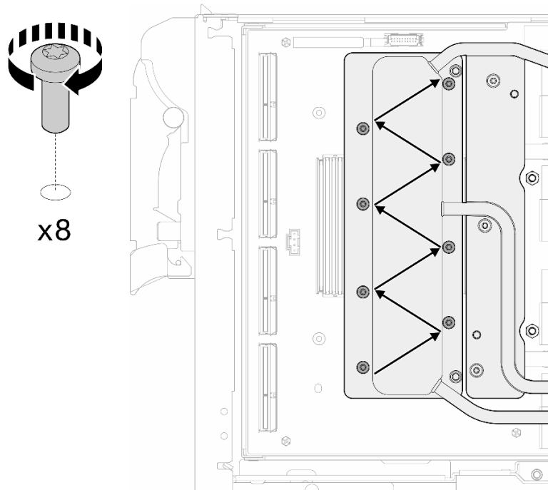
그림 441. 네트워크 카드 나사 설치
