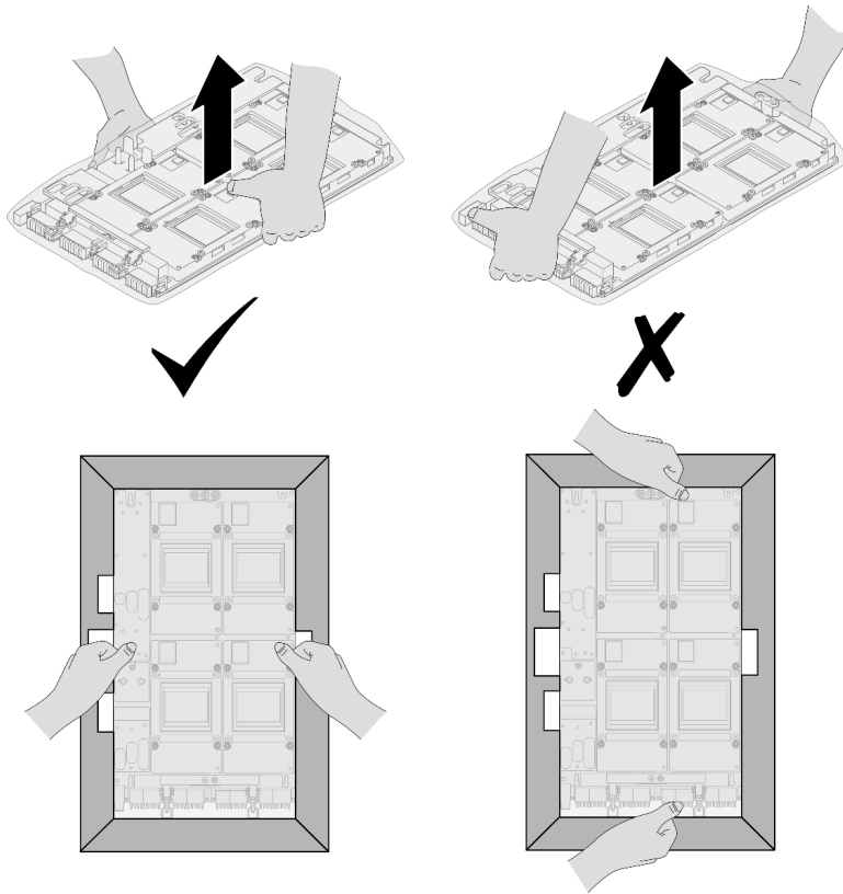
그림 372. 패키지 상자에서 GPU 보드 어셈블리 제거
