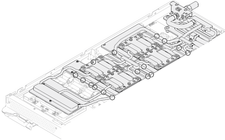
그림 423. GPU 냉각판 분리를 위한 노치
