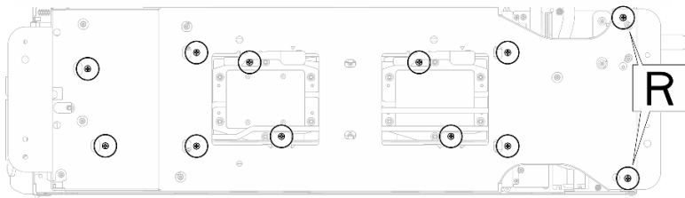
그림 201. 워터 루프 캐리어 나사 풀기
