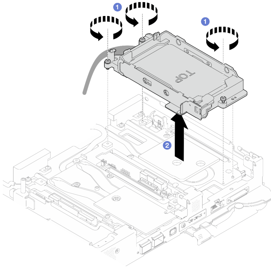
그림 88. 7mm 드라이브 케이지 어셈블리 1개 제거
