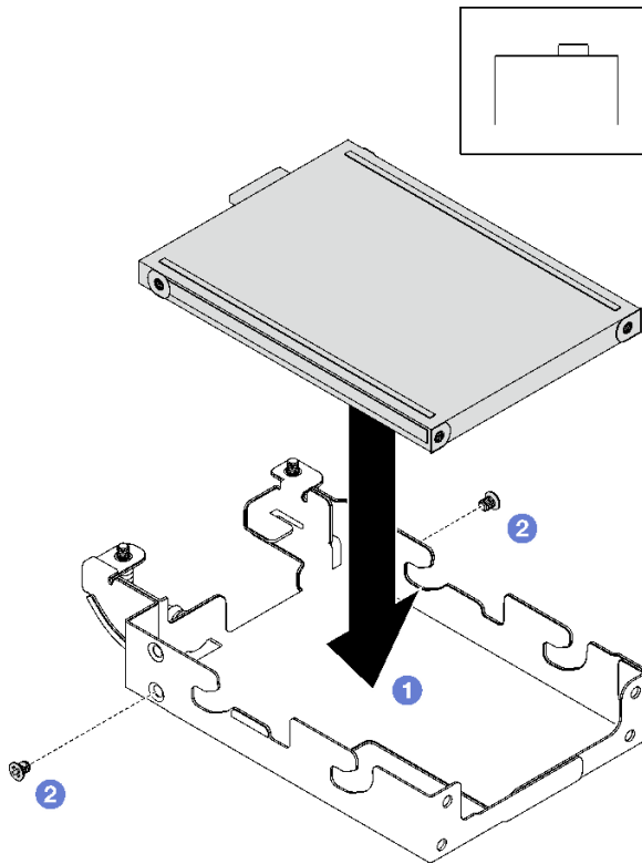
그림 130. 상단 E3.s 드라이브 설치
