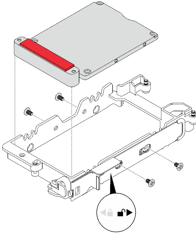
그림 94. 전도판 제거
