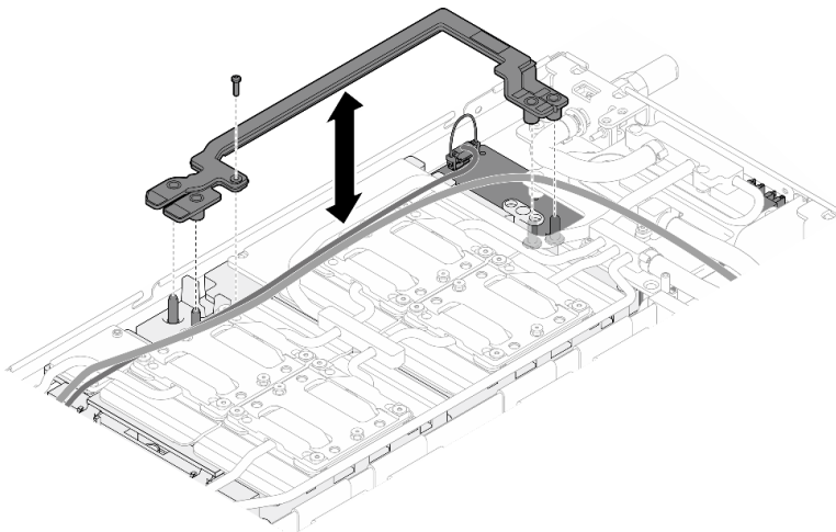
그림 311. 버스 바 설치
