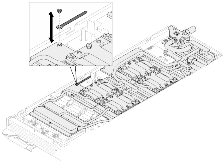
그림 67. 케이블 타이 설치
