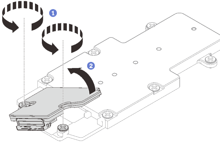
그림 144. M.2 백플레인 어셈블리 분해
