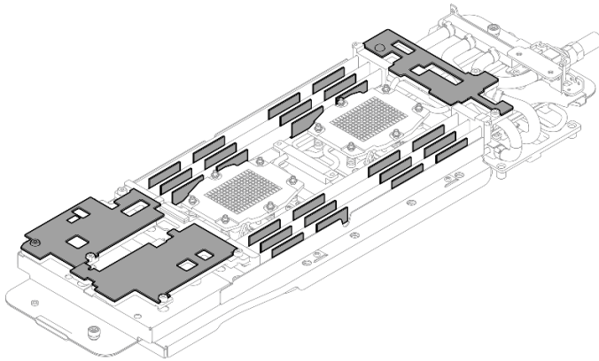
그림 44. 워터 루프 하단 겹 패드(컴퓨팅 노드 쪽)
