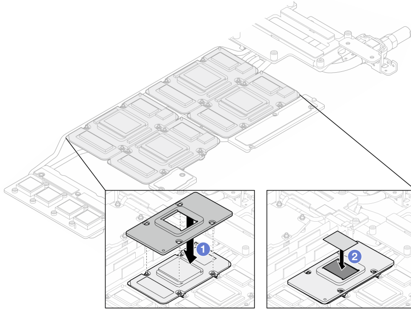
그림 401. 워터 루프 GPU 냉각판 PCM 교체(GPU 노드)
