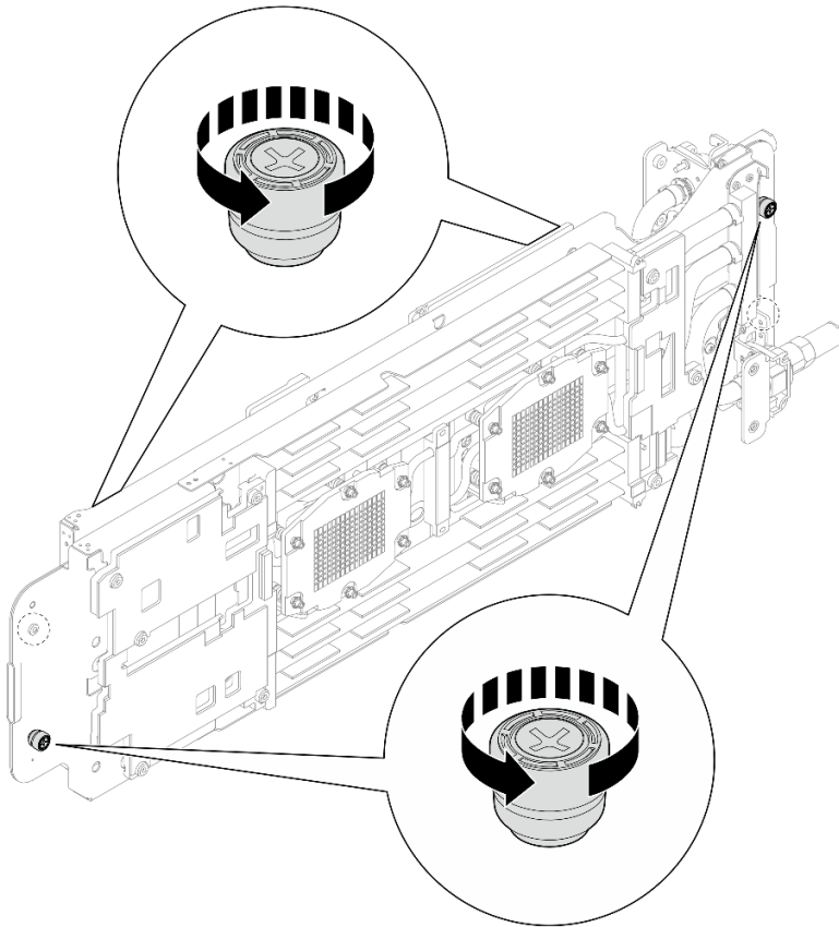
그림 42. 워터 루프 캐리어 고정 나비 나사 풀기
