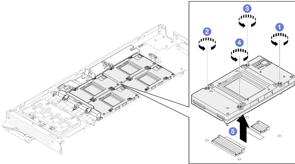
그림 336. GPU 제거
