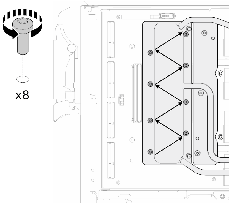
그림 16. 네트워크 카드 나사 제거
