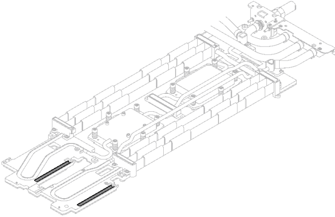
그림 257. 워터 루프 갭 패드(상단)
