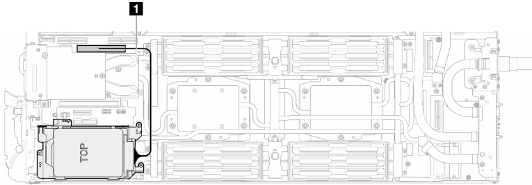
그림 87. 드라이브 케이블 연결 해제
