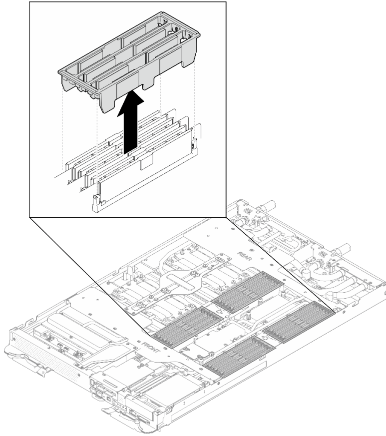
그림 154. DIMM 덮개 제거
