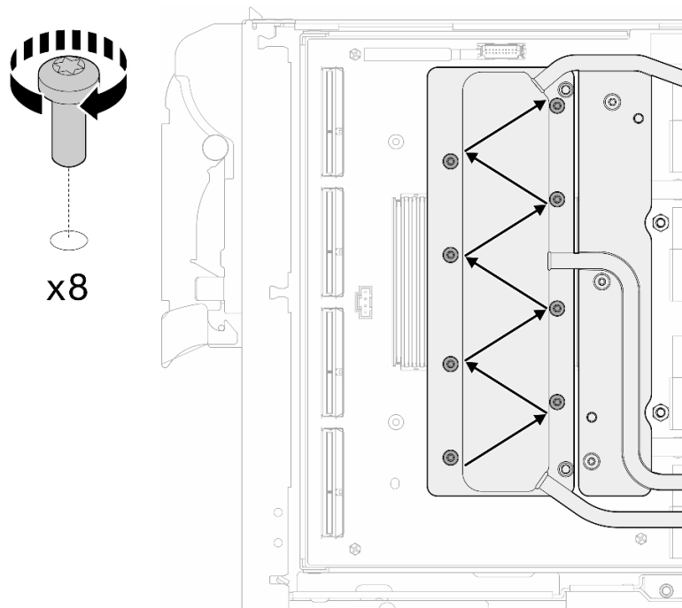
그림 347. 네트워크 카드 나사 설치
