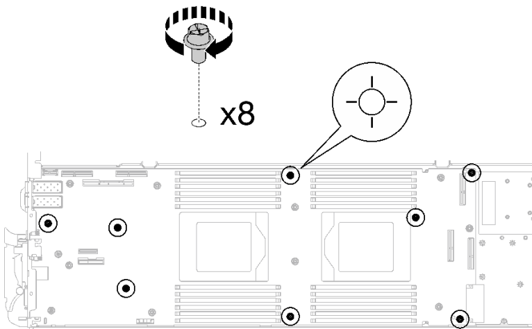
그림 272. 시스템 보드 나사 제거
