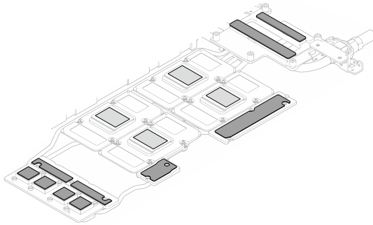
그림 47. 워터 루프 퍼티 패드 교체(GPU 노트)
