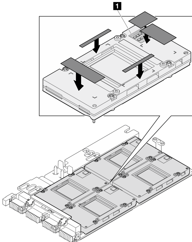
그림 48. GPU 퍼티 패드 교체
