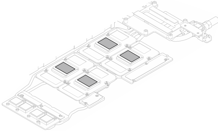
그림 428. 모든 GPU에서 PCM 닦아 내기
