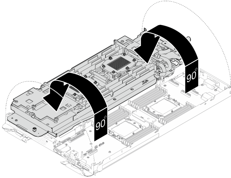
그림 192. 워터 루프 접기
