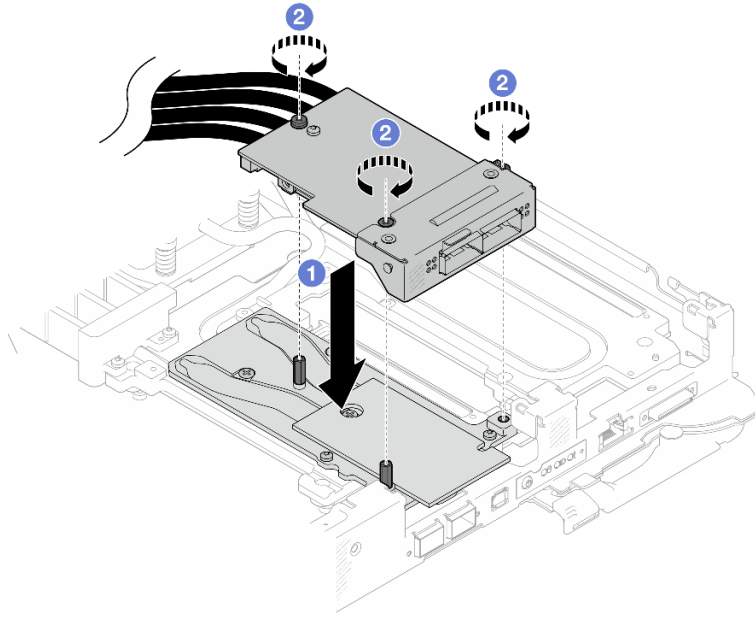
그림 176. OSFP 모듈 설치
