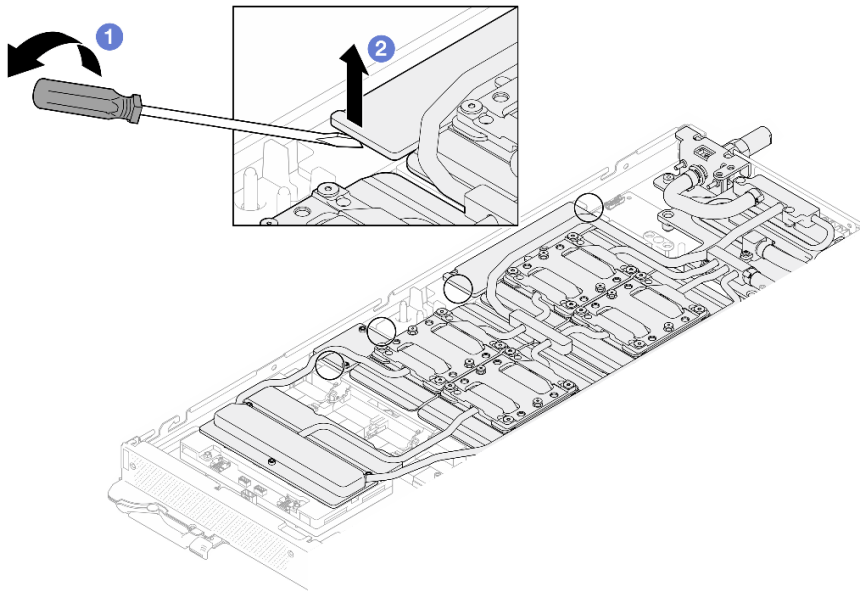
그림 422. 전면 및 후면 MISC 전도판을 GPU 보드에서 분리
