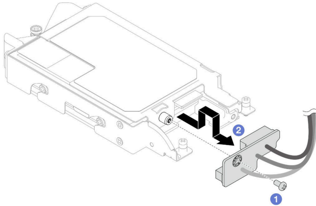
그림 126. E3.s 드라이브 케이블 종단 백플레인 제거
