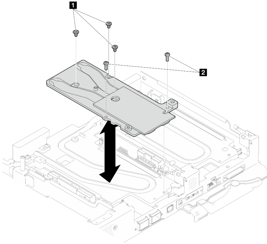
그림 242. OSFP 모듈 전도판 제거
