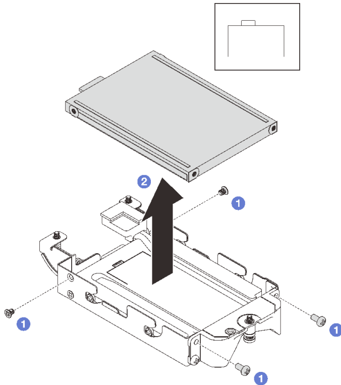
그림 127. 하단 E3.s 드라이브 제거
