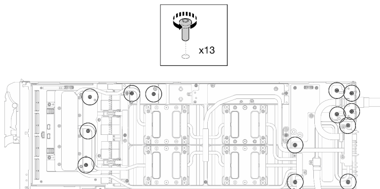
그림 418. 워터 루프 Torx T10 나사 제거(GPU 노드)
