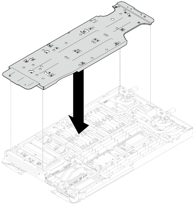
그림 425. 워터 루프 캐리어 설치(GPU 노드)
