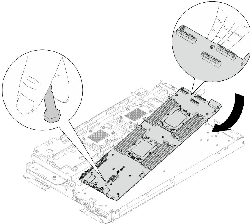
그림 276. 시스템 보드 설치
