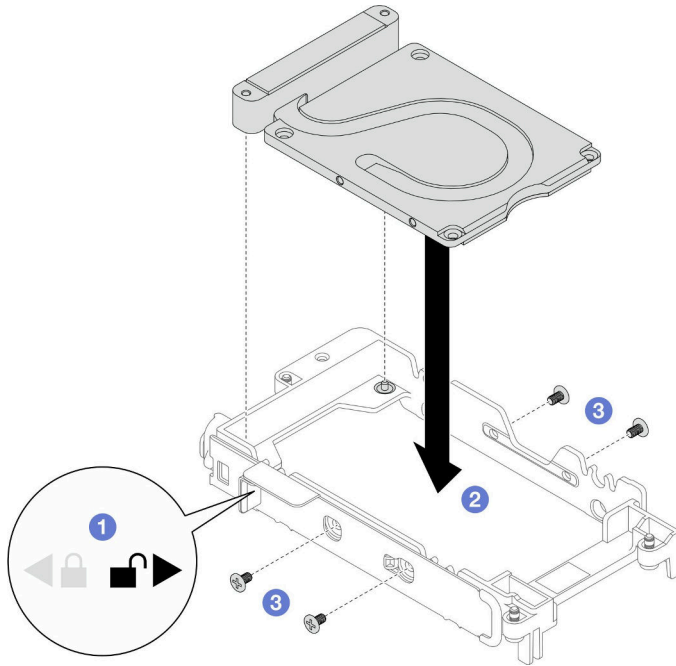
그림 113. 전도판 설치
