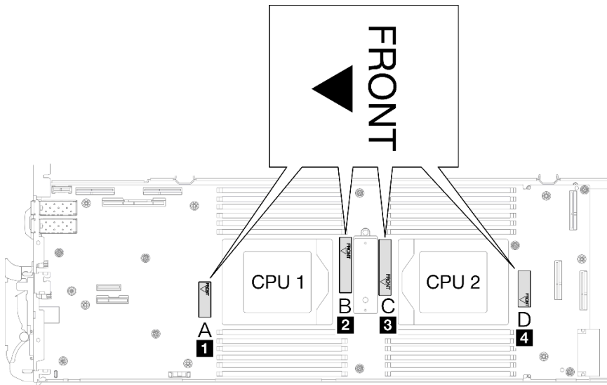
그림 289. 앞면을 가리키는 케이지의 앞면 표시
