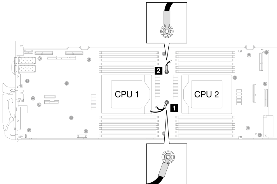
그림 72. 차폐 케이블 1/2 및 차폐 케이블 3을 나사 구멍에 맞추기
