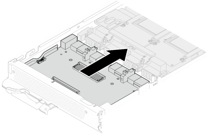
그림 377. GPU 보드에 캐리어 보드 연결.
