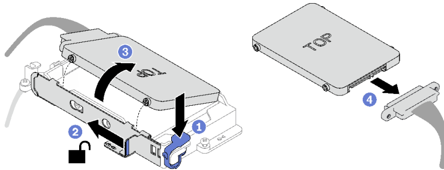
그림 92. 상단 드라이브 제거
