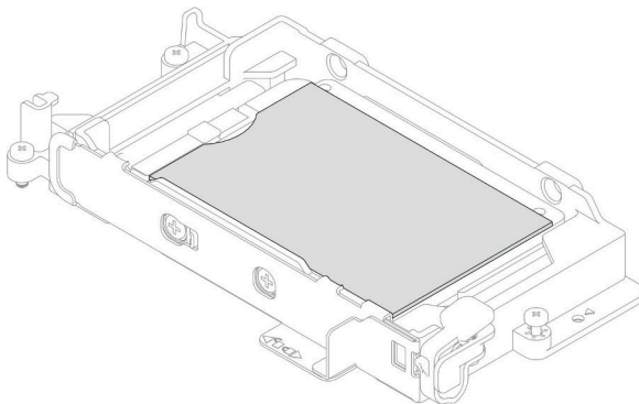
그림 112. 전도판 갭 패드 설치
