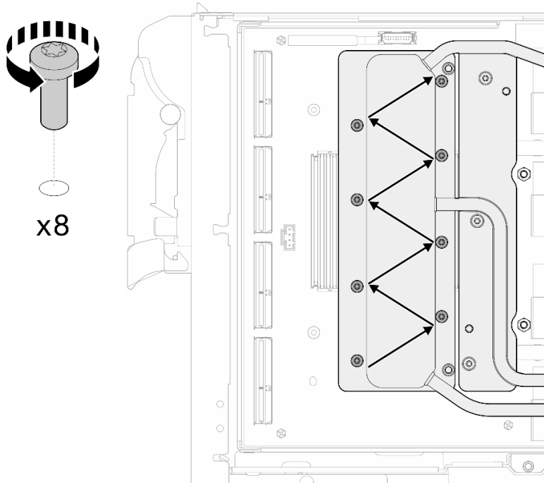
그림 386. 네트워크 카드 나사 제거
