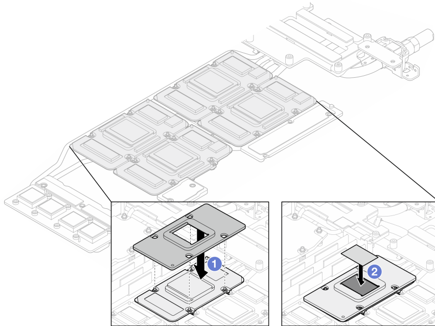
그림 46. 워터 루프 GPU 냉각판 PCM 교체(GPU 노드)
