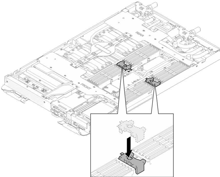
그림 85. DIMM 콤 설치
