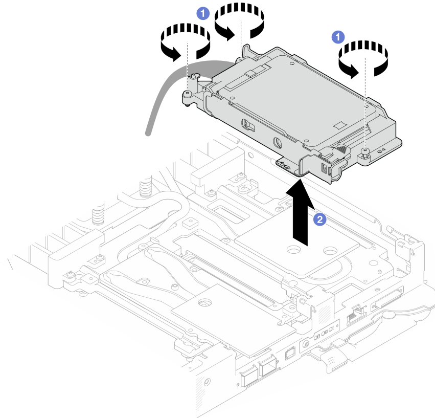
그림 108. 7mm NVMe 드라이브 케이징 어셈블리 제거
