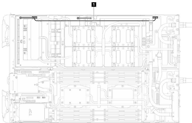
그림 446. 캐리어 보드 전원 케이블 연결
