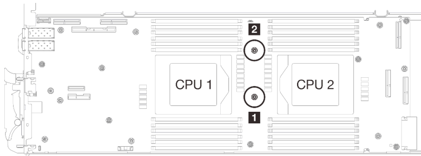
그림 278. 차폐 케이블 1/2 및 3의 나사 구멍 위치
