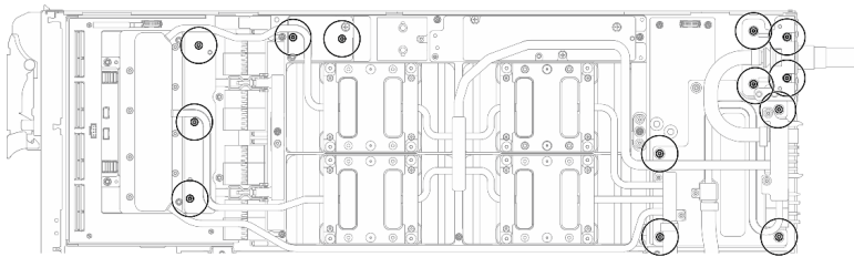
그림 443. 워터 루프 Torx T10 나사 설치(GPU 노드)
