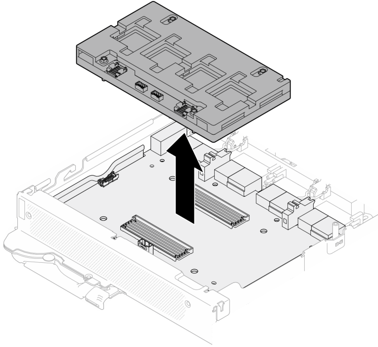
그림 431. 네트워크 보드 제거
