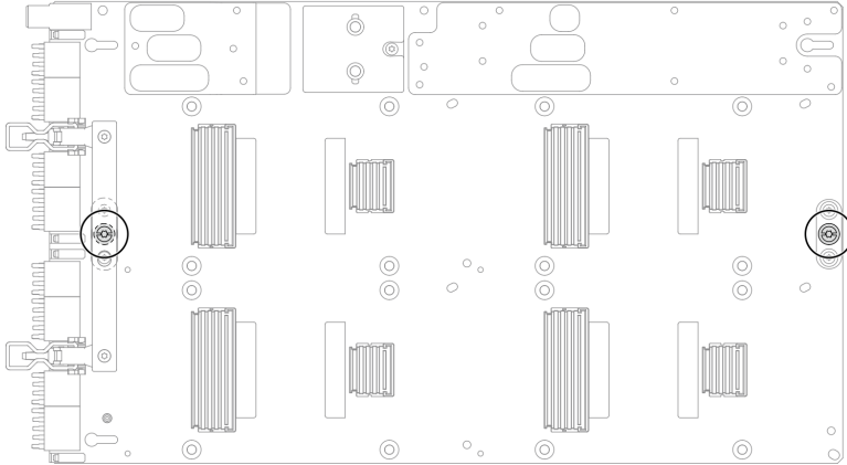
그림 357. GPU 보드 T15 나사 제거
