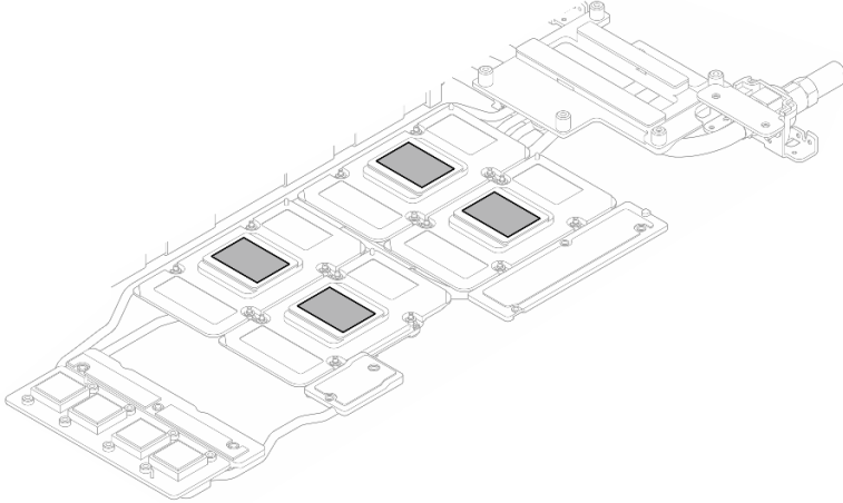
그림 24. 모든 GPU에서 PCM 닦아 내기
