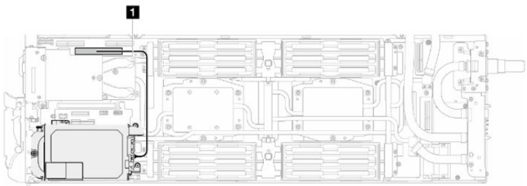
그림 181. E3.S 드라이브 케이블 연결
