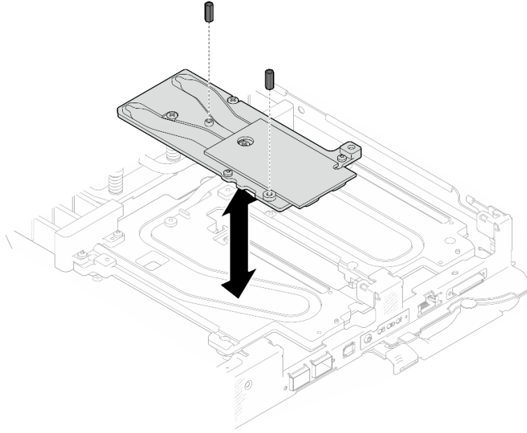
그림 269. OSFP 모듈 전도판 육각 나사 설치
