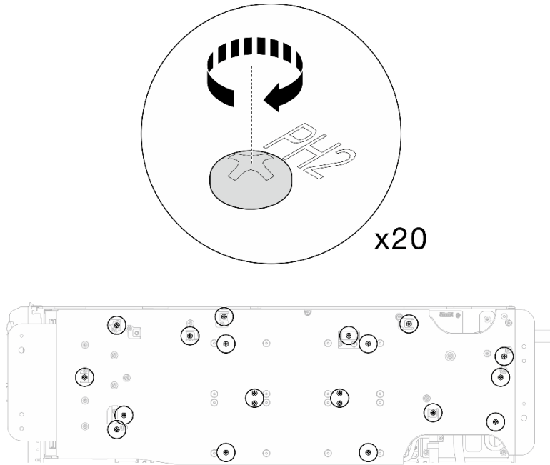
그림 426. 워터 루프 나사 및 빠른 연결 나사 제거(GPU 노드)
