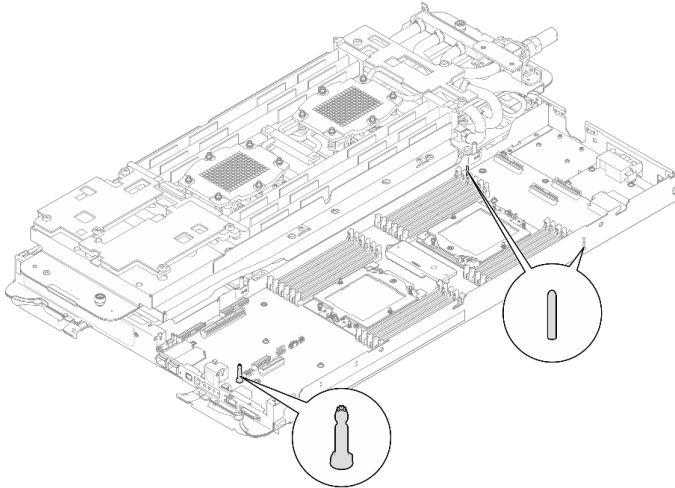
그림 199. 컴퓨팅 노드의 가이드 핀
