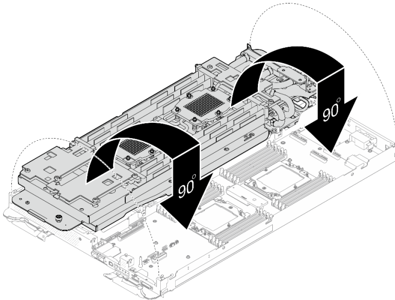
그림 260. 워터 루프 설치
