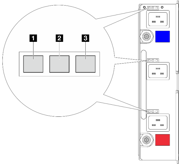
그림 460. DWC 전원 공급 장치 LED
