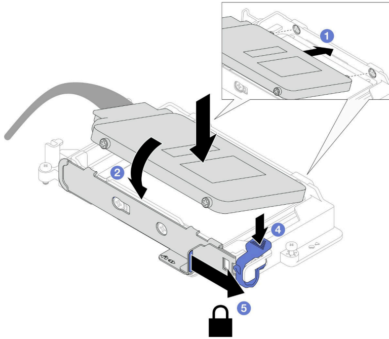
그림 115. 위쪽 드라이브 설치
