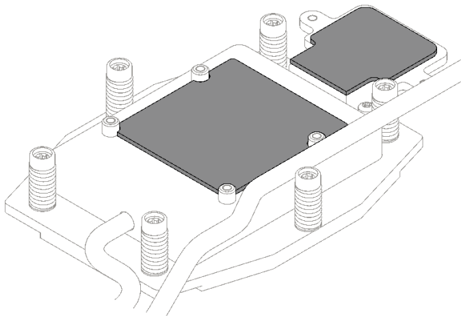
그림 149. 프로세서 냉각판 및 M.2 냉각판의 퍼티 패드
