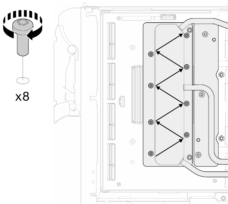
그림 408. 네트워크 카드 나사 설치
