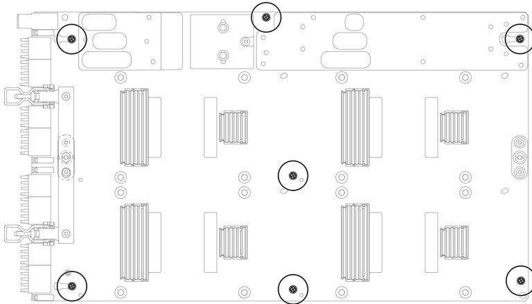
그림 362. GPU 보드에 M3 나사 설치
