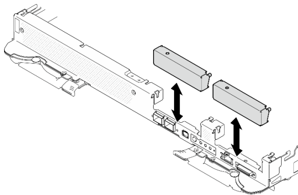
그림 90. 빈 베젤 필터 제거
