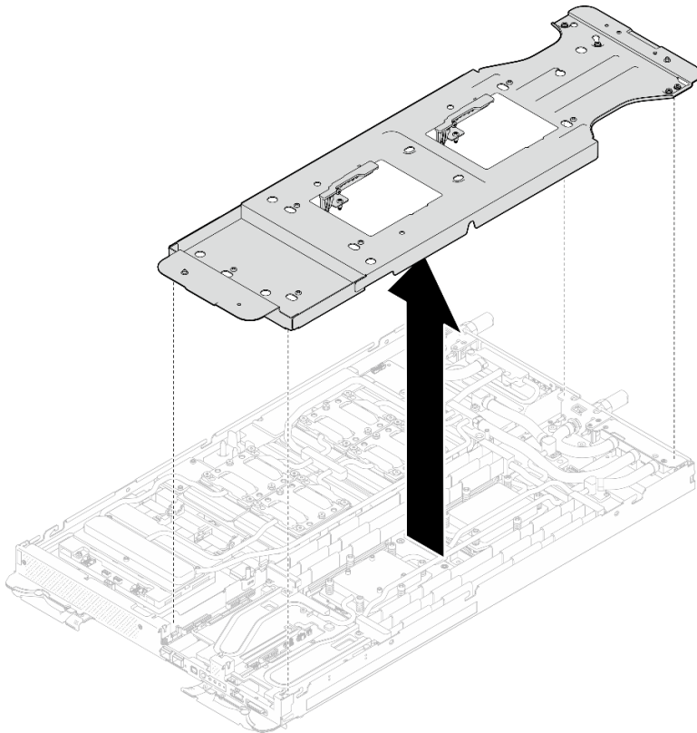
그림 202. 워터 루프 캐리어 제거(컴퓨팅 노드)
