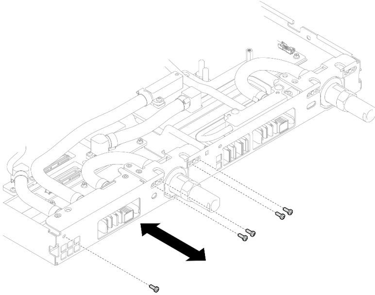
그림 237. 퀵 커넥트 나사 설치(컴퓨팅 노드)
