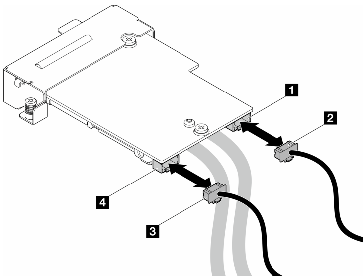
그림 173. OSFP 모듈 전원 케이블 제거
