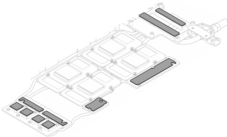
그림 429. 워터 루프에서 퍼티 패드 닦아 내기
