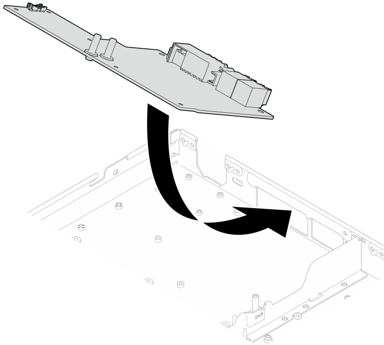
그림 399. GPU 전원 분배 보드 설치
