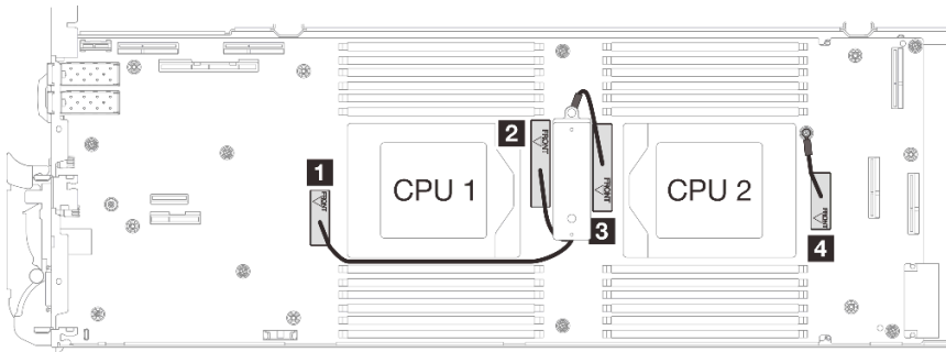
그림 292. 차폐 케이스의 케이블 배선
