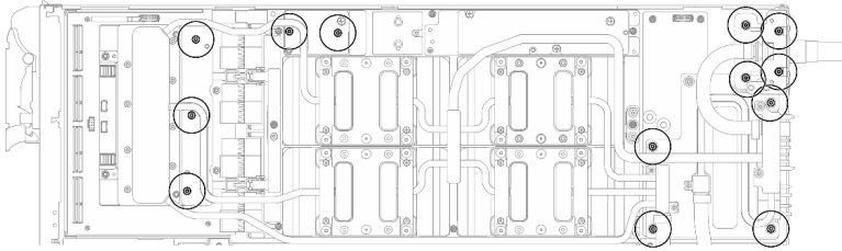
그림 384. 워터 루프 Torx T10 나사 제거(GPU 노트)
