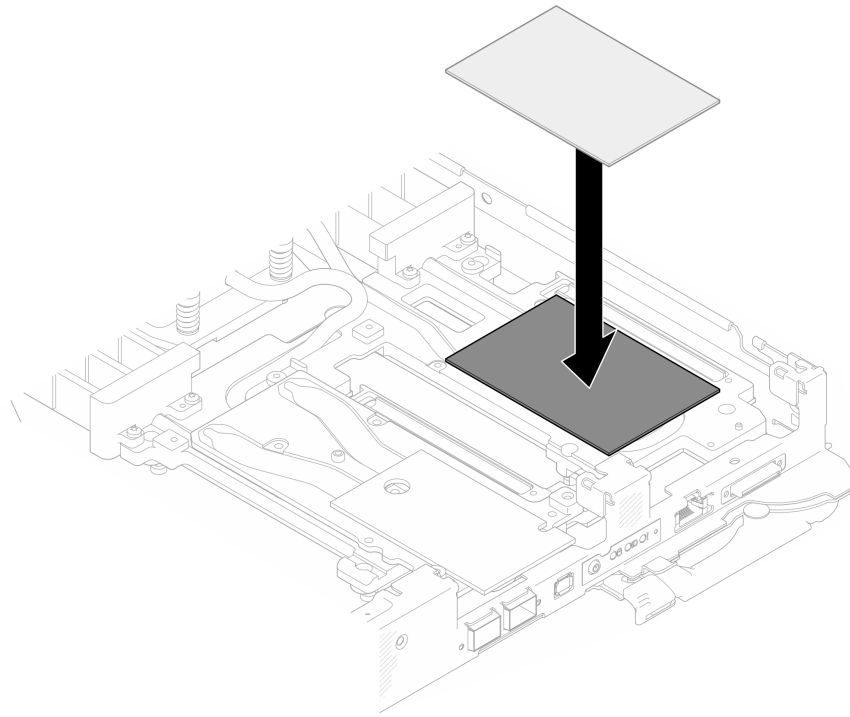
그림 139. 갭 패드 교체
