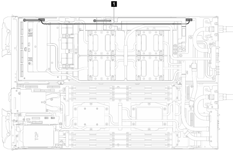
그림 312. 캐리어 보드 전원 케이블 제거
