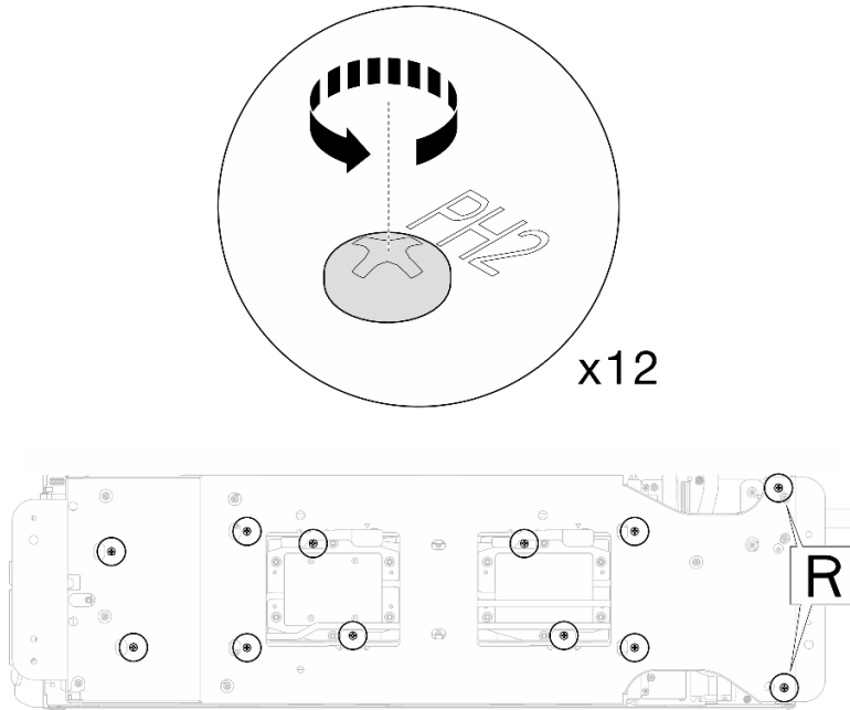
그림 261. 워터 루프 캐리어 나사 풀기
