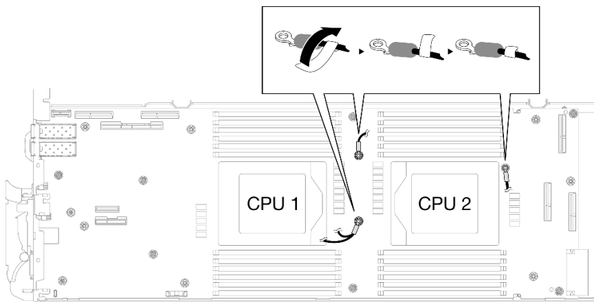
그림 302. 차폐 케이블에 레이블 감기
