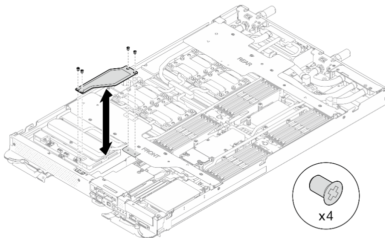
그림 10. 전면 케이블 덮개 설치
