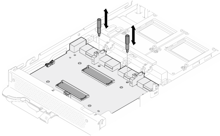
그림 313. 캐리어 보드 스탠드오프 제거
