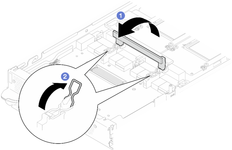
그림 368. 캐리어 보드 분리
