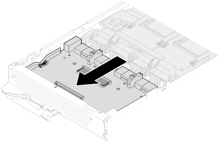
그림 369. GPU 보드에서 캐리어 보드 연결 해제
