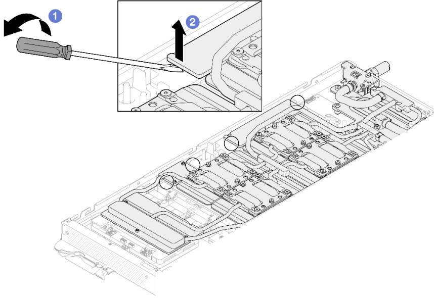
그림 18. 전면 및 후면 MISC 전도판을 GPU 보드에서 분리
