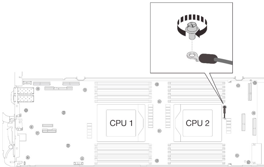
그림 301. 차폐 케이블 4 설치
