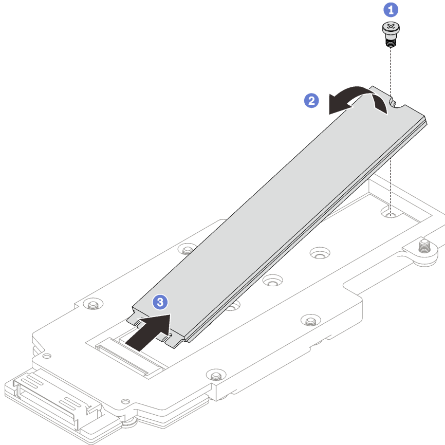
그림 145. M.2 드라이브 제거
