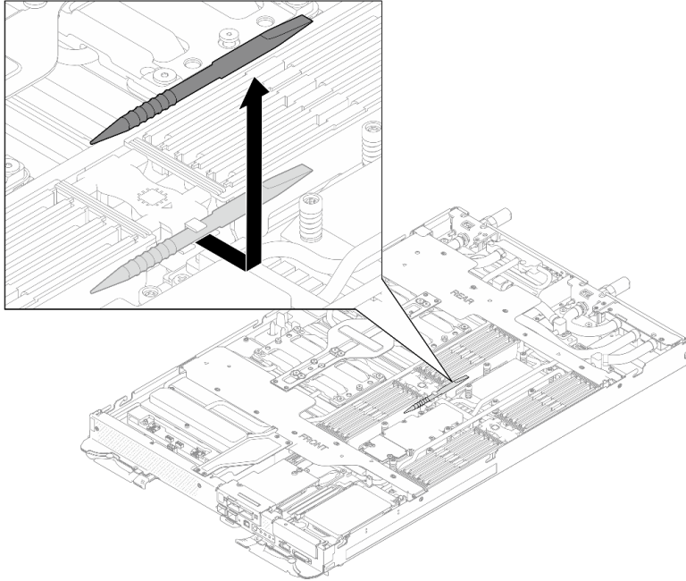
그림 83. 메모리 모듈 도구 제거
