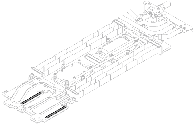
그림 197. 워터 루프 갭 패드(상단)
