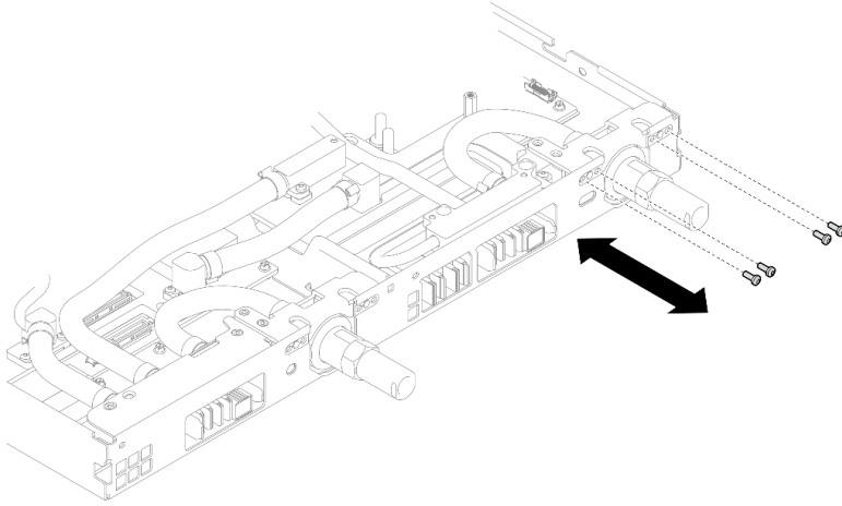
그림 442. 퀵 커넥트 나사 설치(GPU 노드)
