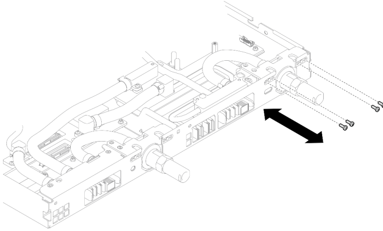
그림 348. 퀵 커넥트 나사 설치(GPU 노드)
