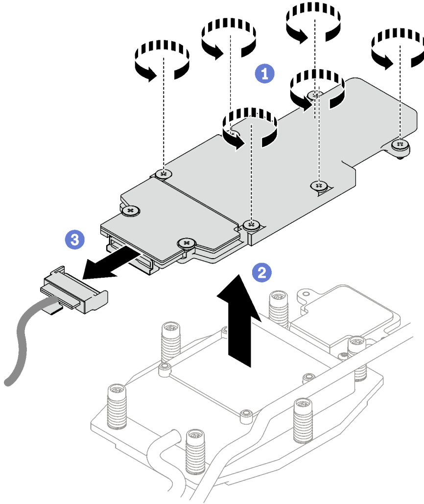
그림 143. M.2 백플레인 어셈블리 제거
