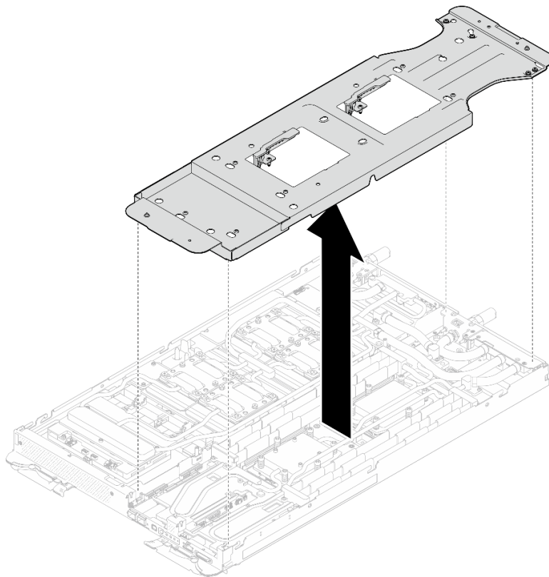
그림 262. 워터 루프 캐리어 제거(컴퓨팅 노드)
