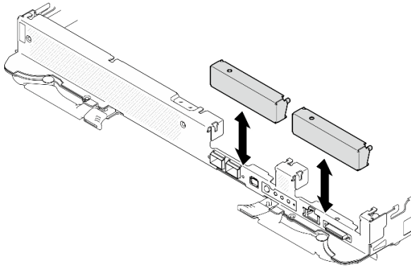
그림 109. 빈 베젤 필터 제거
