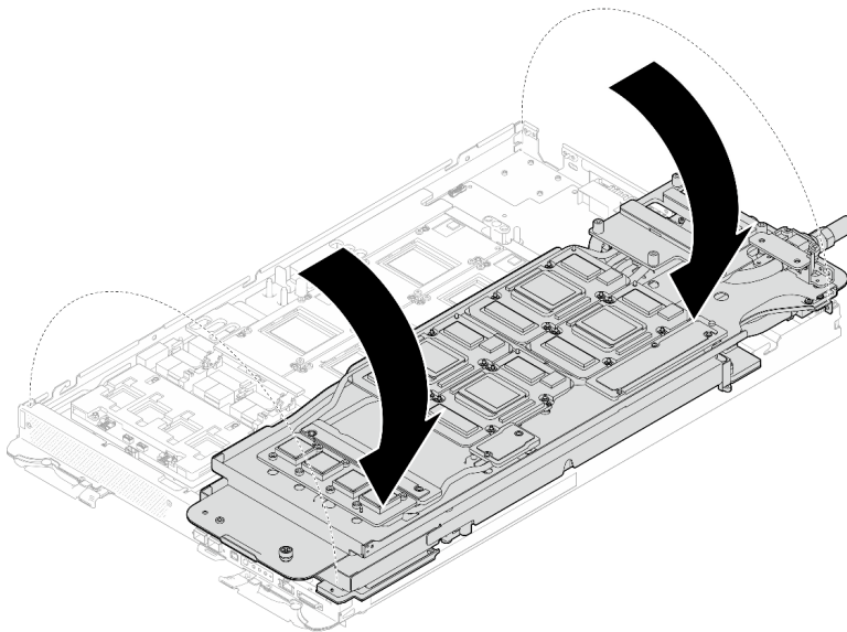
그림 333. GPU 노드 측 워터 루프를 컴퓨팅 노드 측 워터 루프 쪽으로 접기
