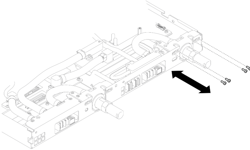
그림 419. 퀵 커넥트 나사 제거(GPU 노드)
