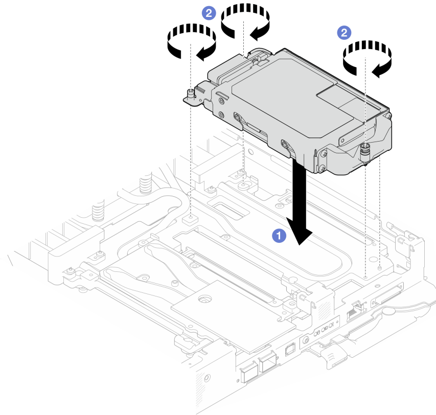
그림 140. E3.S 드라이브 케이지 어셈블리 설치
