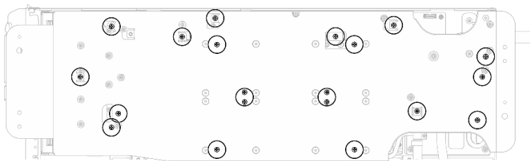
그림 60. 워터 루프 나사 및 킥 커넥트 나사 설치(GPU 노드)
