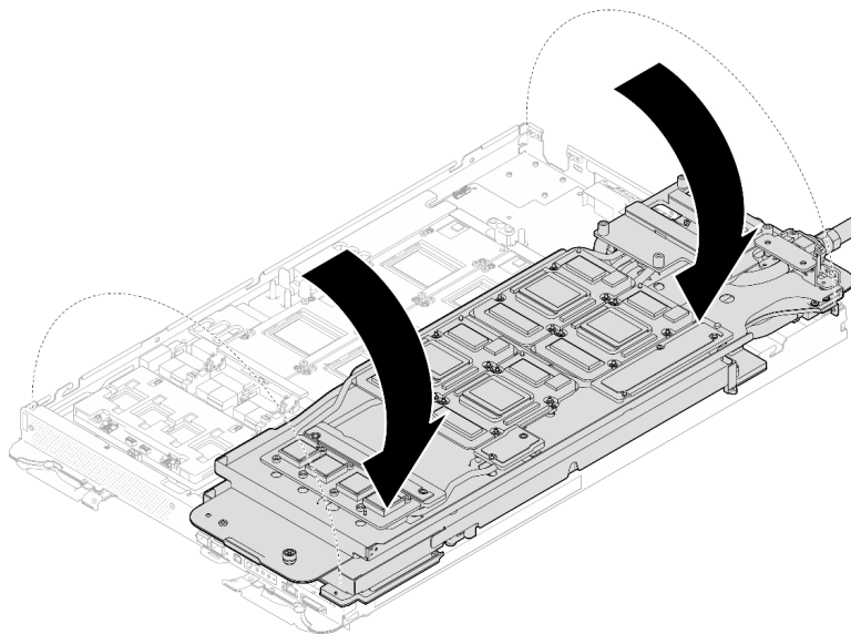
그림 23. GPU 노드 측 워터 루프를 컴퓨팅 노드 측 워터 루프 쪽으로 접기
