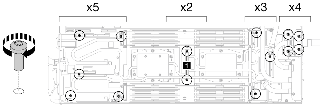
그림 265. 워터 루프 나사 및 퀵 커넥트 나사 설치
