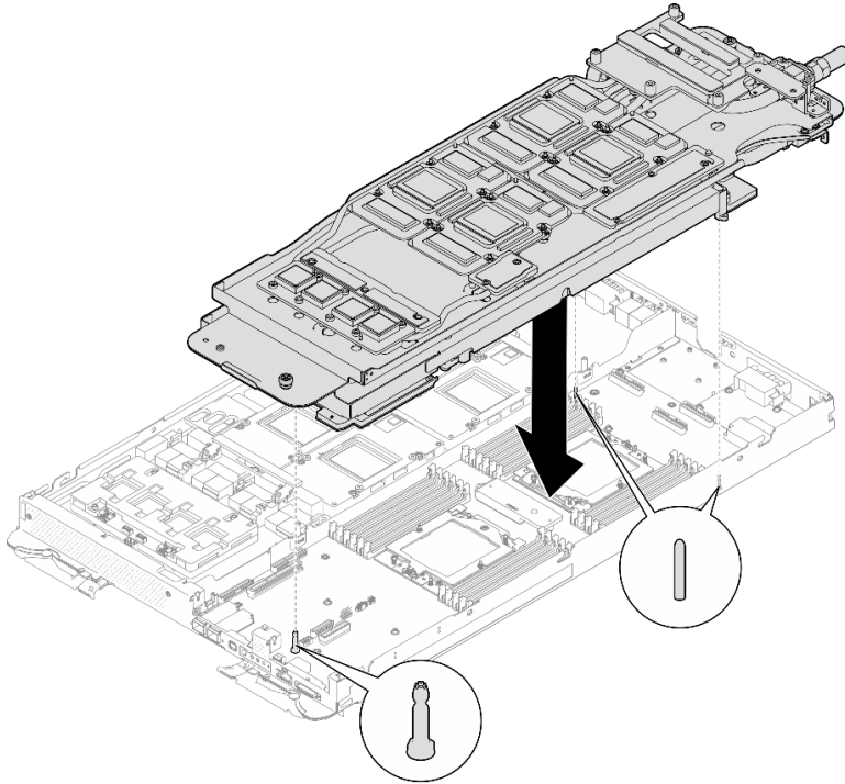
그림 49. 워터 루프 캐리어 설치
