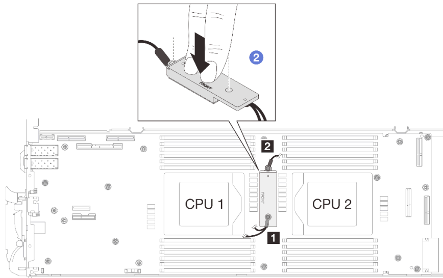
그림 74. VR 전도판 누르기
