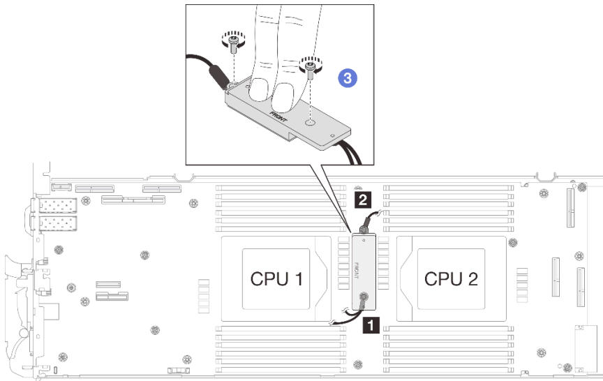
그림 282. 차폐 케이블 1/2 및 3 설치
