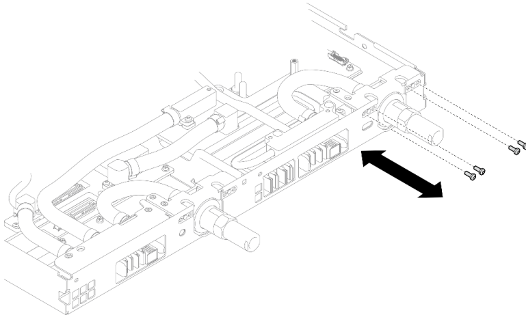
그림 409. 퀵 커넥트 나사 설치(GPU 노드)
