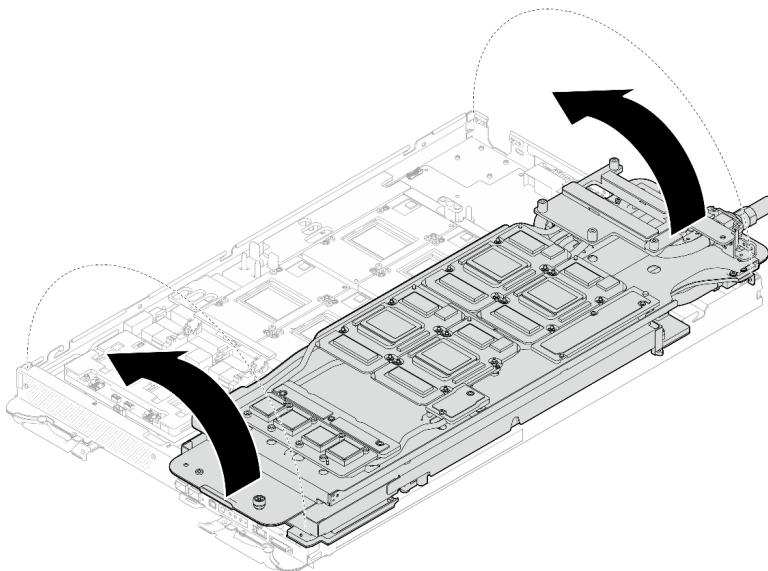
그림 437. 워터 루프를 GPU 노드에 펼치기
