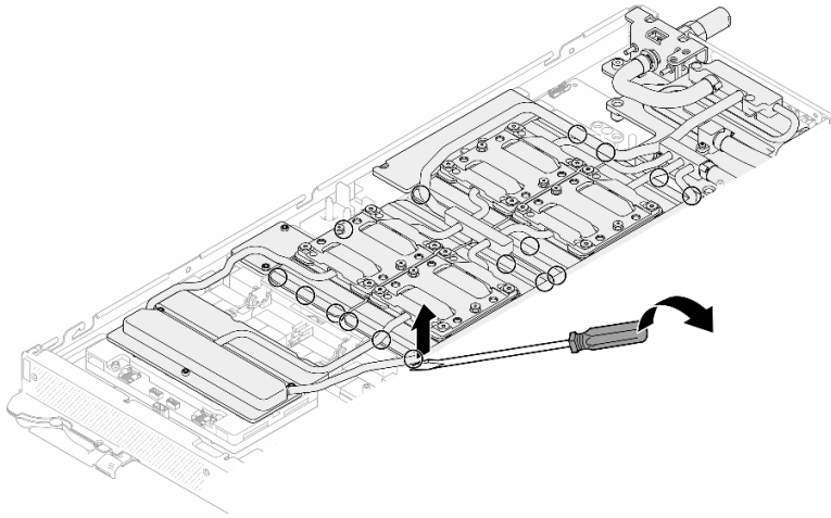
그림 20. GPU에서 GPU 냉각판 분리
