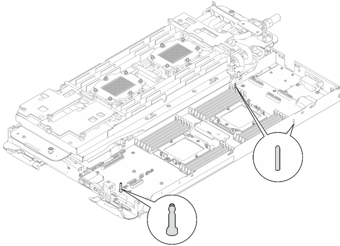
그림 259. 컴퓨팅 노드의 가이드 핀
