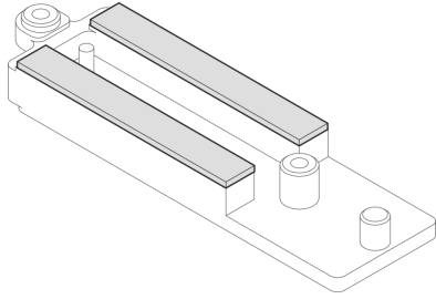
그림 77. VR 전도판 하단의 퍼티 패드
