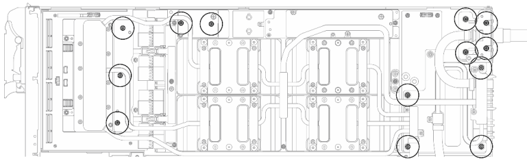
그림 65. 워터 루프 Torx T10 나사 설치(GPU 노드)
