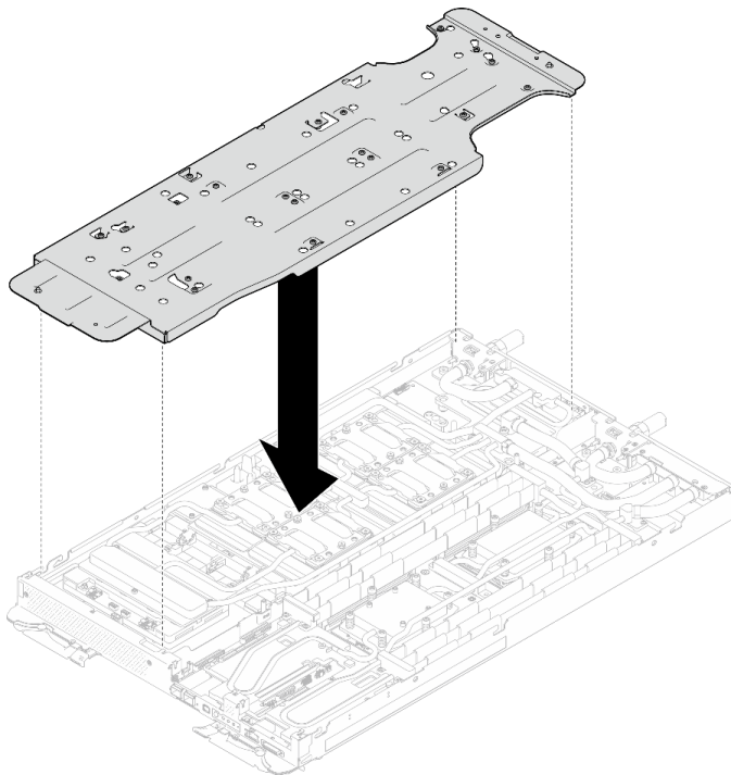
그림 21. 워터 루프 캐리어 설치(GPU 노드)
