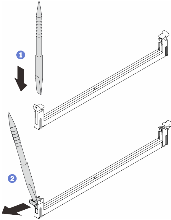
그림 155. 메모리 모듈 제거
