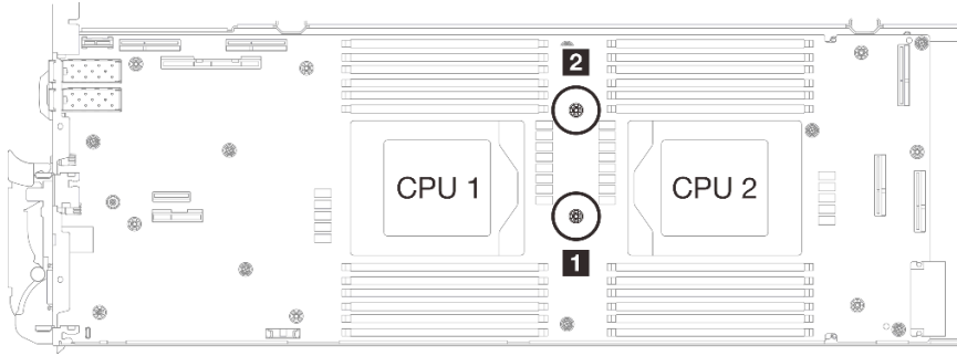
그림 71. 차폐 케이블 1/2 및 3의 나사 구멍 위치
