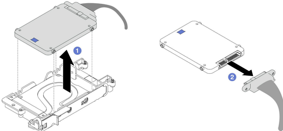
그림 111. 하단 드라이브 제거
