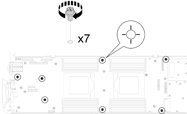
그림 303. 시스템 보드 나사 설치
