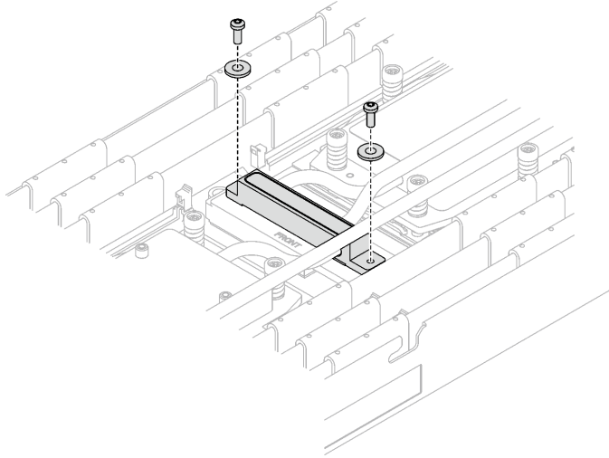
그림 264. 와셔가 있는 VR 냉각판 나사
