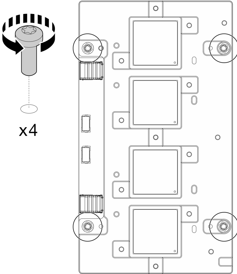
그림 430. 네트워크 보드 나사 제거
