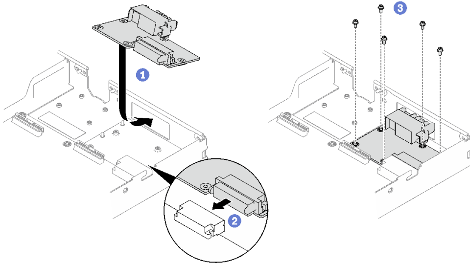
그림 194. 전원 분배 보드 설치
