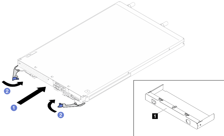
그림 4. 트레이 설치
