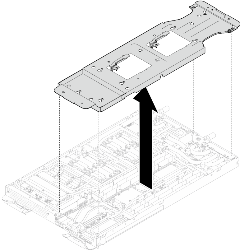
그림 52. 워터 루프 캐리어 제거(컴퓨팅 노드)
