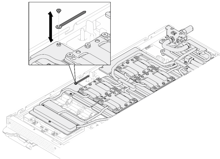
그림 445. 케이블 타이 설치
