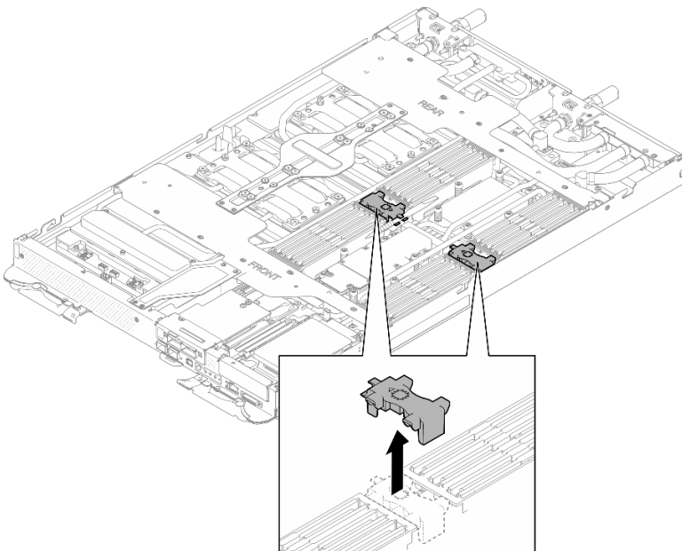
그림 84. DIMM 콤 제거
