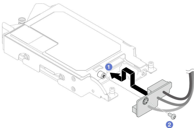
그림 135. E3.s 케이블 종단 백플레인 설치
