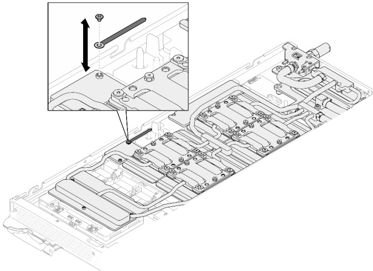
그림 416. 케이블 타이 제거
