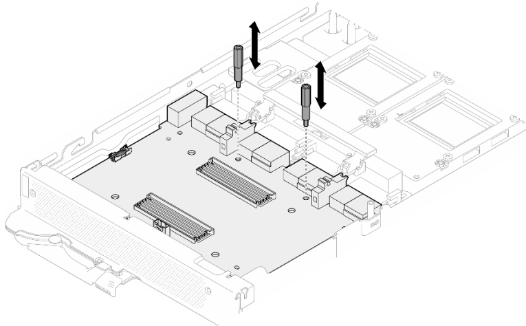
그림 318. 캐리어 보드 스탠드오프 설치
