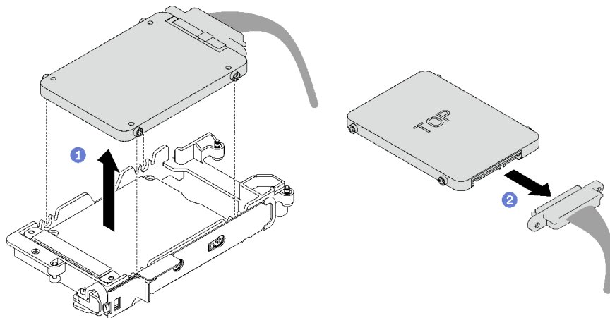
그림 93. 하단 드라이브 제거
