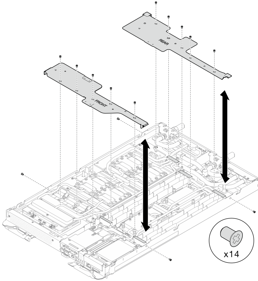
그림 9. 전면 및 후면 십자형 브레이스 설치
