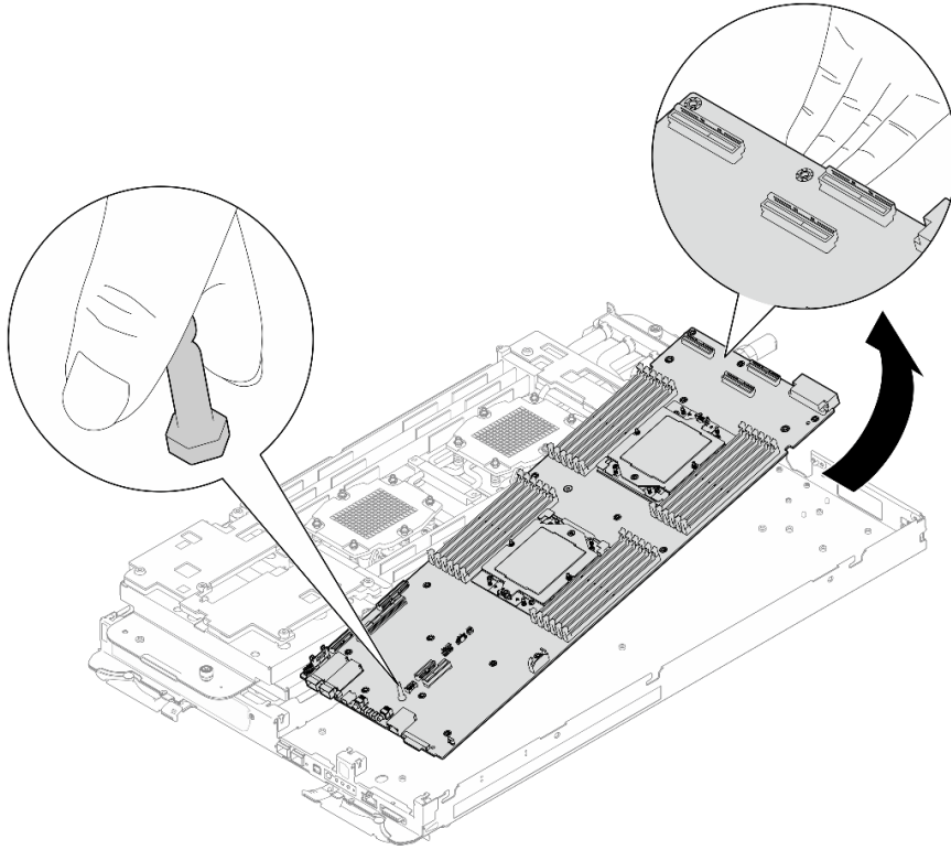
그림 273. 시스템 보드 제거
