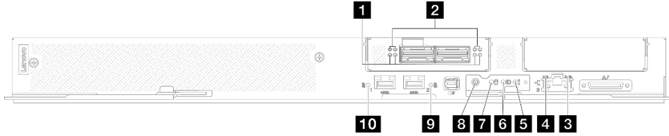
그림 457. SD665-N V3 트레이 앞면 LED
