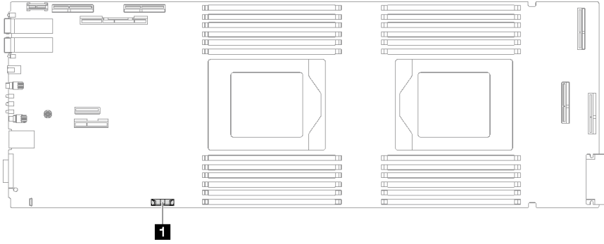
그림 79. CMOS 배터리 위치
