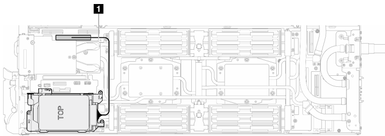
그림 120. 드라이브 케이지 케이블 연결
