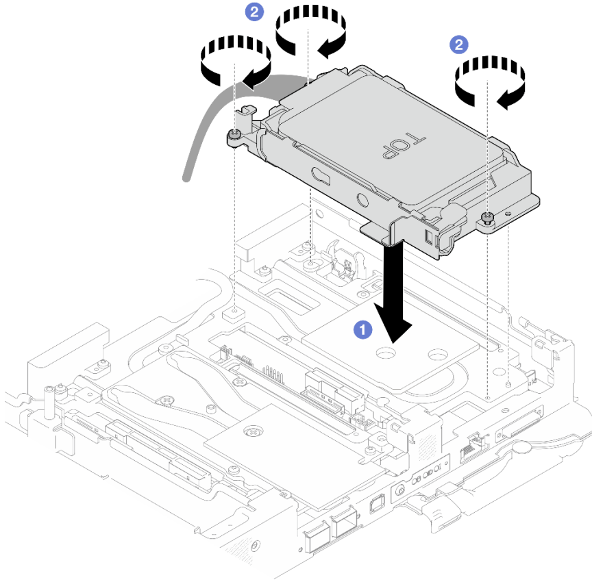
그림 105. 7mm 드라이브 케이지 어셈블리 2개 설치
