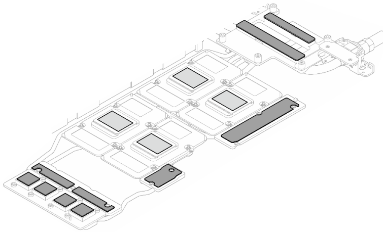
그림 435. 워터 루프 퍼티 패드 교체(GPU 노드)
