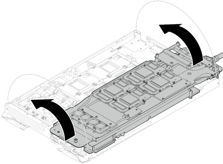
그림 26. GPU 노드 워터 루프를 GPU 노드로 뒤집기
