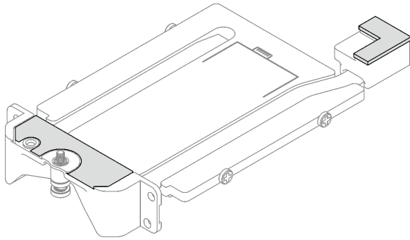
그림 132. 전도판 퍼티 패드 교체
