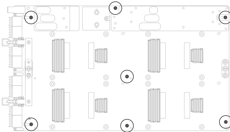
그림 356. GPU 보드 M3 나사 제거
