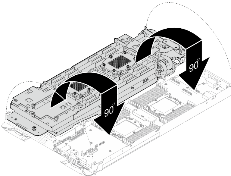
그림 200. 워터 루프 설치
