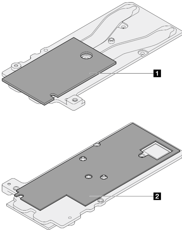
그림 238. OSFP 모듈 전도판 퍼티 패드 교체
