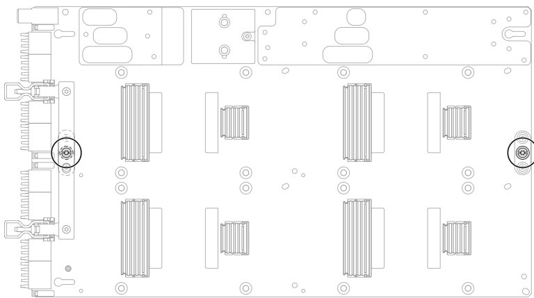
그림 363. GPU 보드에 T15 나사 설치
