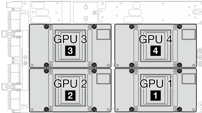
그림 337. GPU 번호
