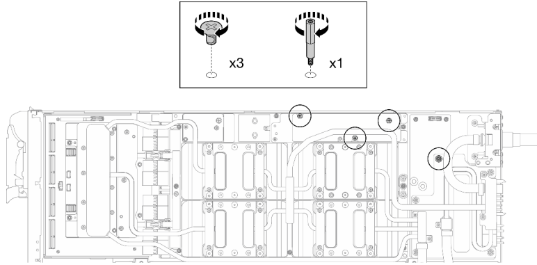
그림 350. 워터 루프 육각 및 PH1 나사 설치(GPU 노드)
