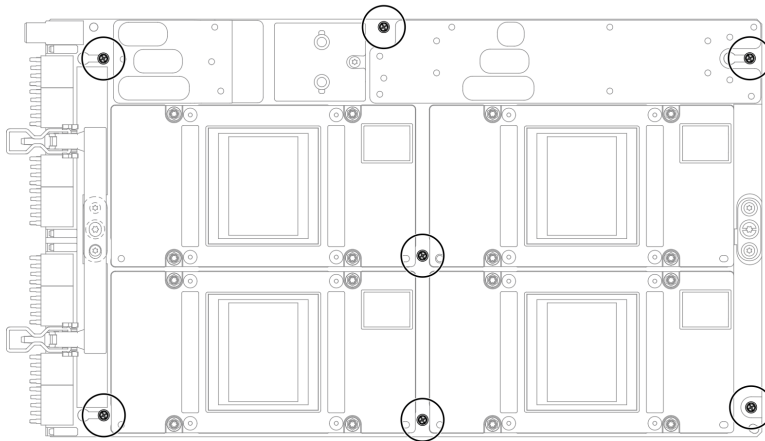
그림 370. GPU 보드 어셈블리 M3 나사 제거
