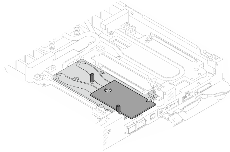
그림 174. OSFP 모듈의 퍼티 패드 교체
