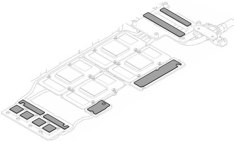
그림 335. 워터 루프에서 퍼티 패드 닦아 내기
