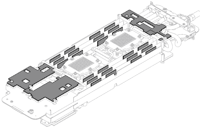
그림 196. 워터 루프 갭 패드(하단)
