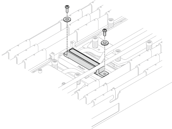
그림 235. 와셔가 있는 VR 냉각판 나사
