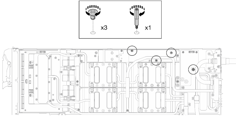
그림 411. 워터 루프 육각 및 PH1 나사 설치(GPU 노드)
