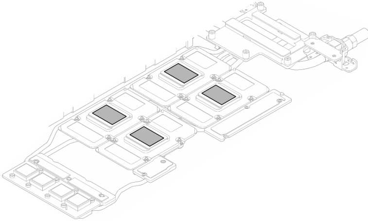
그림 334. 모든 GPU에서 PCM 닦아 내기
