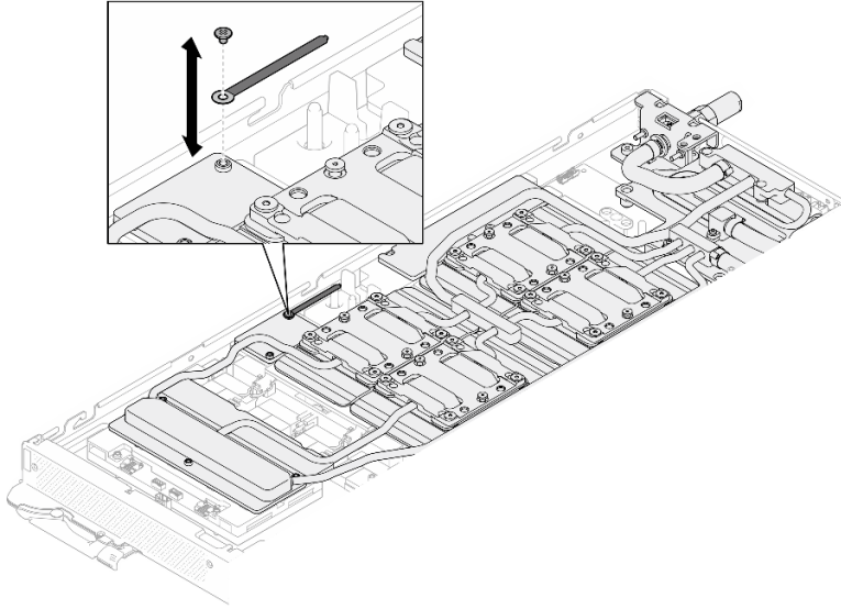
그림 382. 케이블 타이 제거
