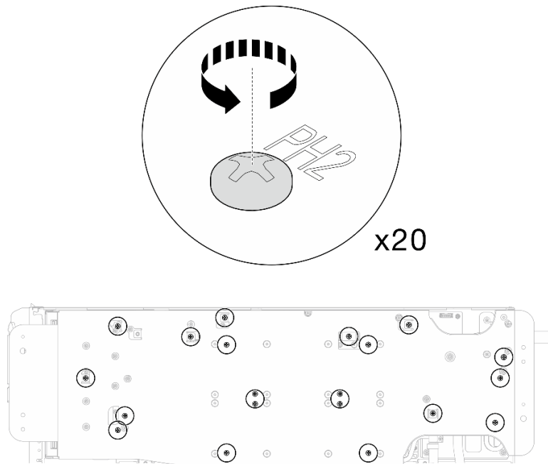
그림 405. 워터 루프 나사 및 퀵 커넥트 나사 설치(GPU 노드)
