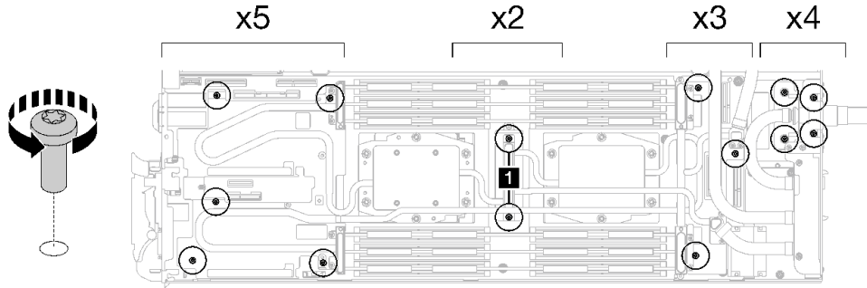
그림 215. 워터 루프 나사 제거
