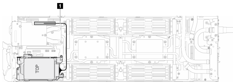
그림 106. 드라이브 케이지 케이블 연결
