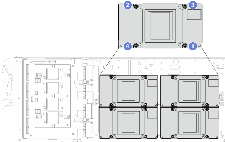
그림 339. GPU 나사 조임 순서
