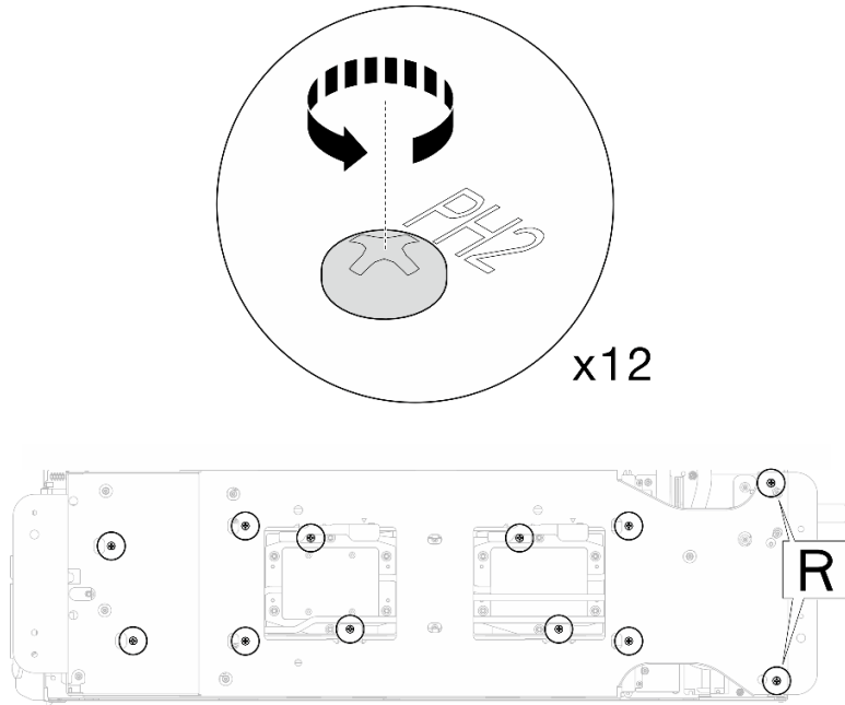
그림 219. 워터 루프 캐리어 나사 설치(컴퓨팅 노드)
