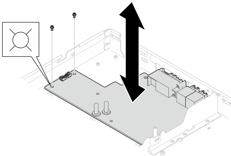
그림 400. GPU 전원 분배 보드 나사 설치
