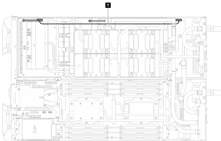
그림 319. 캐리어 보드 전원 케이블 연결
