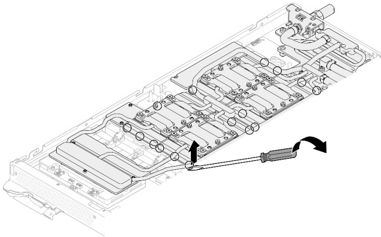
그림 424. GPU에서 GPU 냉각판 분리
