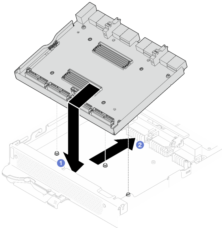
그림 316. 캐리어 보드 설치
