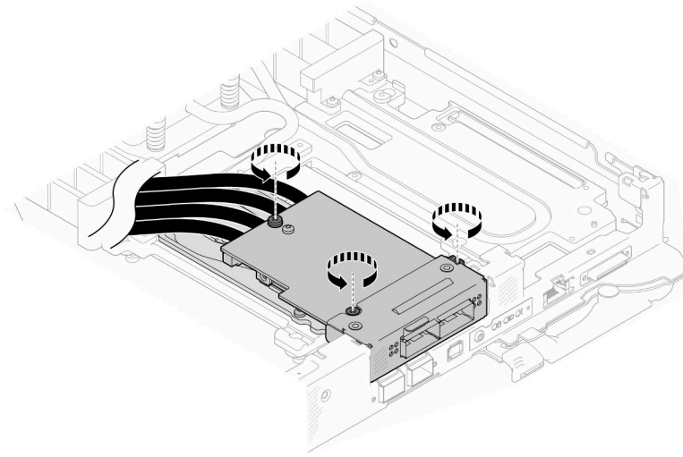
그림 171. OSFP 모듈 제거
