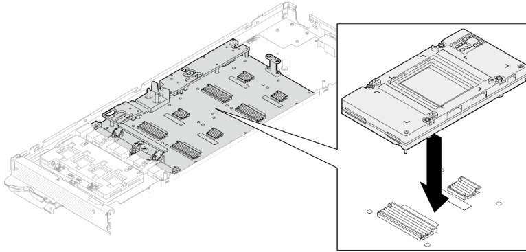
그림 338. GPU 설치
