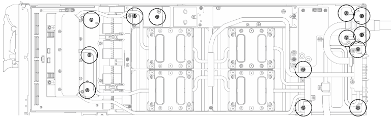
그림 349. 워터 루프 Torx T10 나사 설치(GPU 노드)
