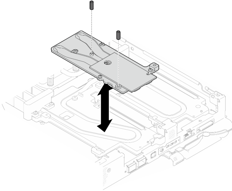
그림 241. OSFP 모듈 전도판 육각 나사 제거
