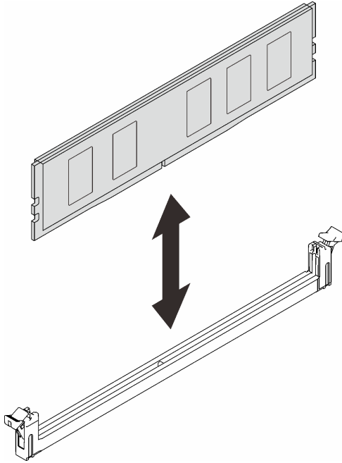
그림 163. 메모리 모듈 설치
