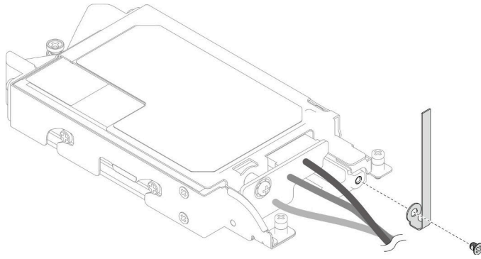
그림 136. 케이블 타이 설치
