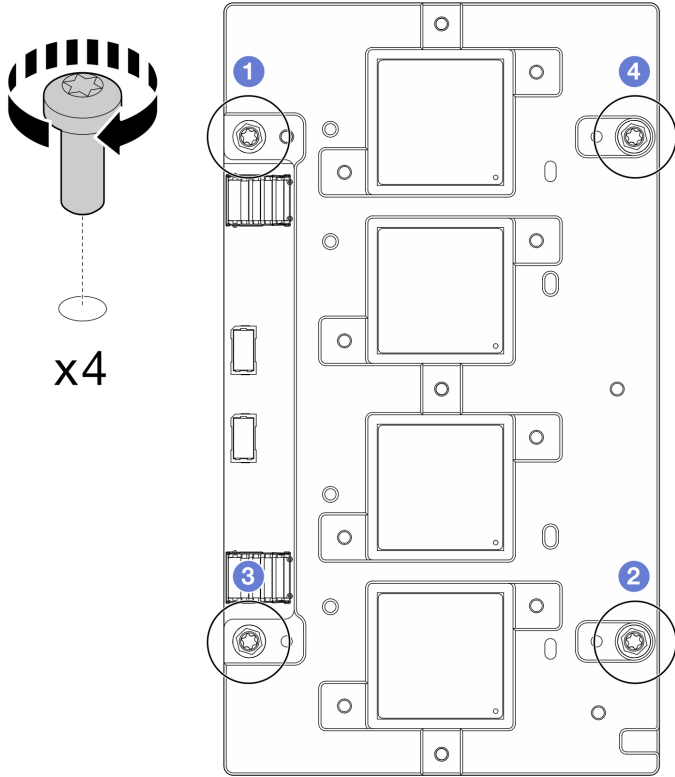
그림 433. 네트워크 보드 나사 설치
