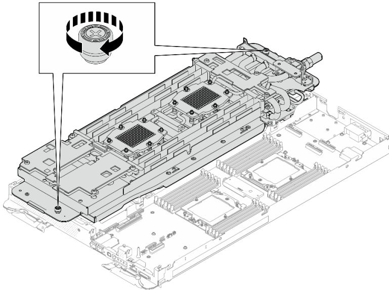
그림 38. 고정 나비 나사 조이기
