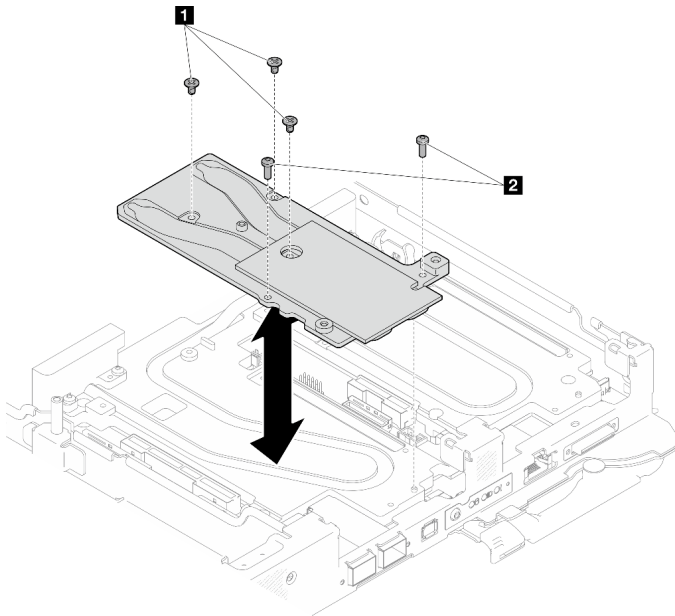
그림 58. OSFP 모듈 전도판 설치
