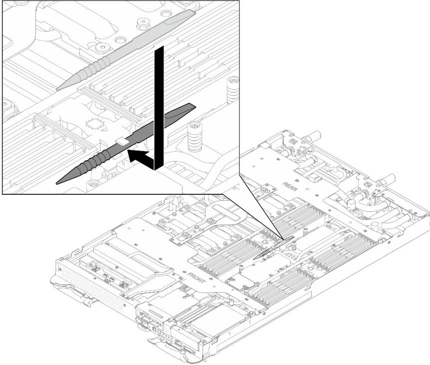
그림 158. 메모리 모듈 도구
