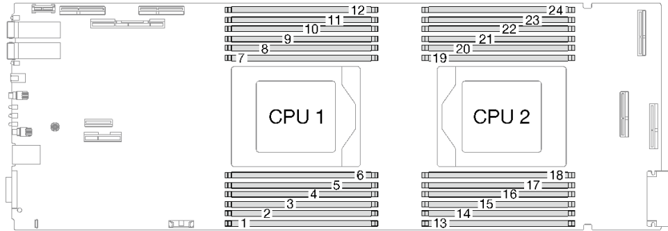
그림 1. 메모리 모듈 및 프로세서 레이아웃
