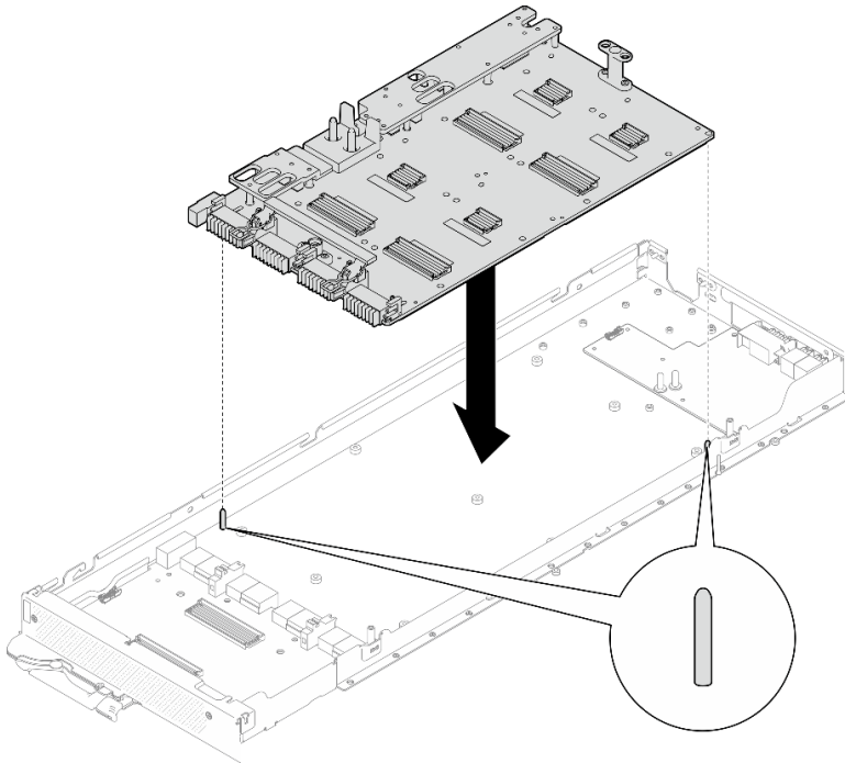
그림 361. GPU 보드 설치
