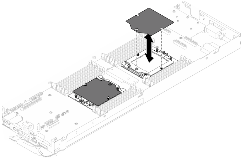
그림 253. 프로세서 소켓 보호 필름 설치
