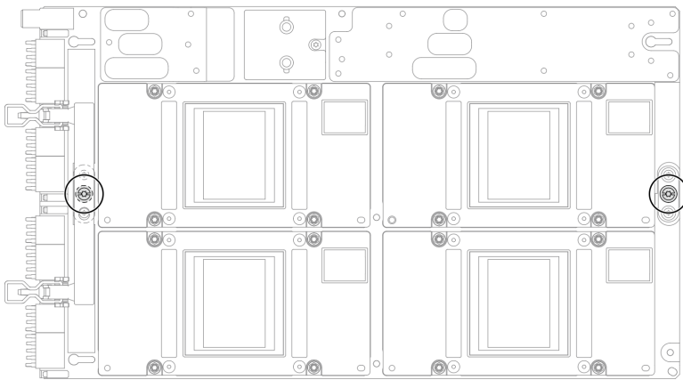
그림 376. GPU 보드 어셈블리에 T15 나사 설치
