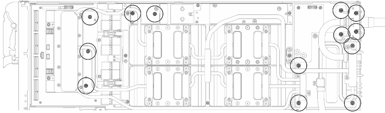
그림 14. 워터 루프 Torx T10 나사 제거(GPU 노드)
