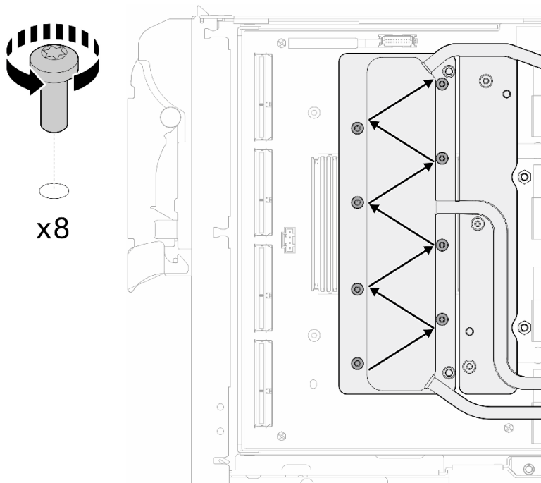
그림 420. 네트워크 카드 나사 제거
