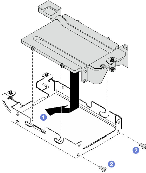
그림 133. E3.s 드라이브 전도판 설치
