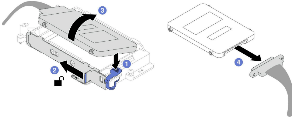
그림 110. 상단 드라이브 제거(7mm NVMe)
