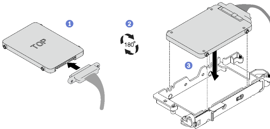
그림 95. 7mm 드라이브 설치
