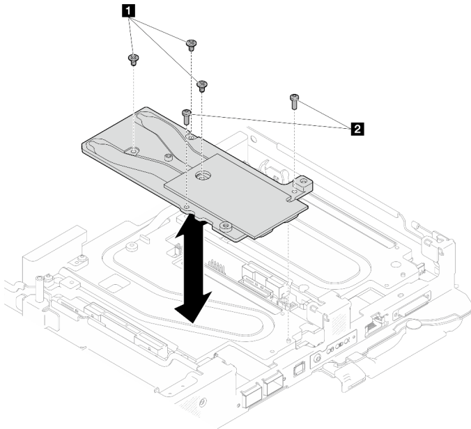
그림 239. OSFP 모듈 전도판 설치
