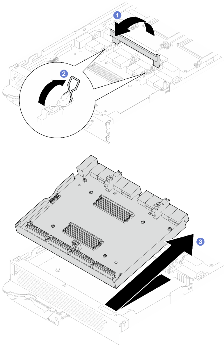
그림 314. 캐리어 보드 제거
