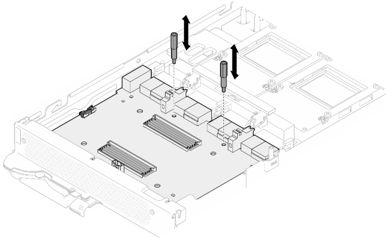
그림 366. 캐리어 보드 스탠드오프 설치
