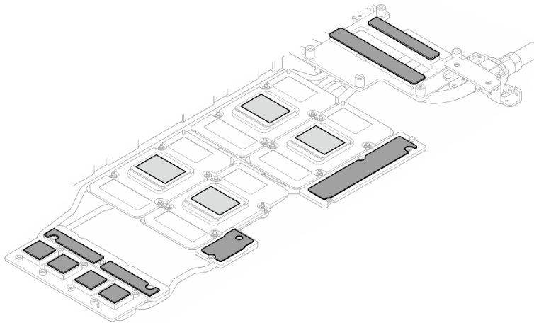
그림 402. 워터 루프 퍼티 패드 교체(GPU 노드)
