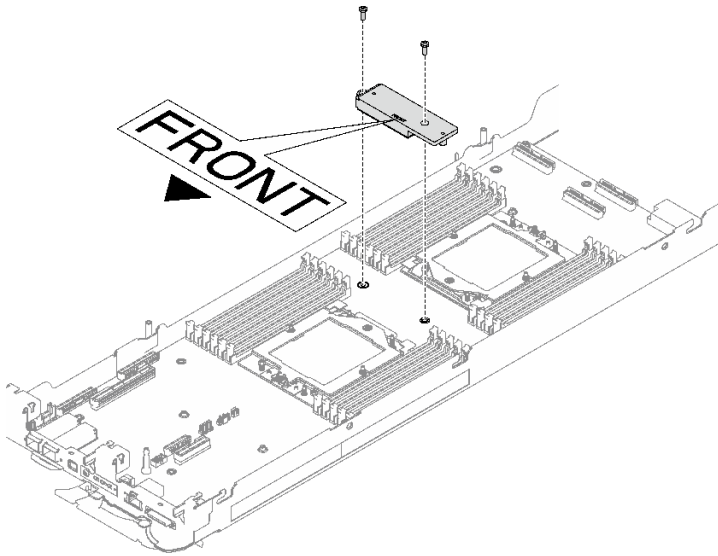
그림 271. VR 전도판 제거
