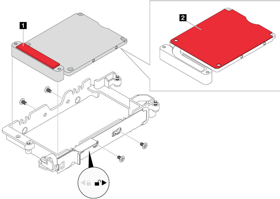
그림 97. 전도판 설치
