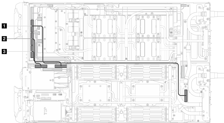
그림 179. 프로세서 2개 구성 - MCIO 2, MCIO 3 및 MCIO 4 케이블을 GPU 노드에 연결
