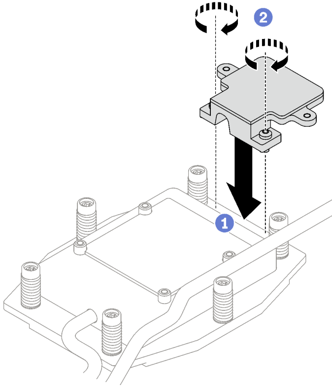
그림 148. M.2 백플레인 냉각판 설치
