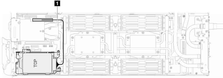
그림 107. 드라이브 케이블 연결 해제
