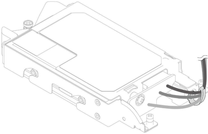
그림 124. 케이블 타이에서 케이블 분리
