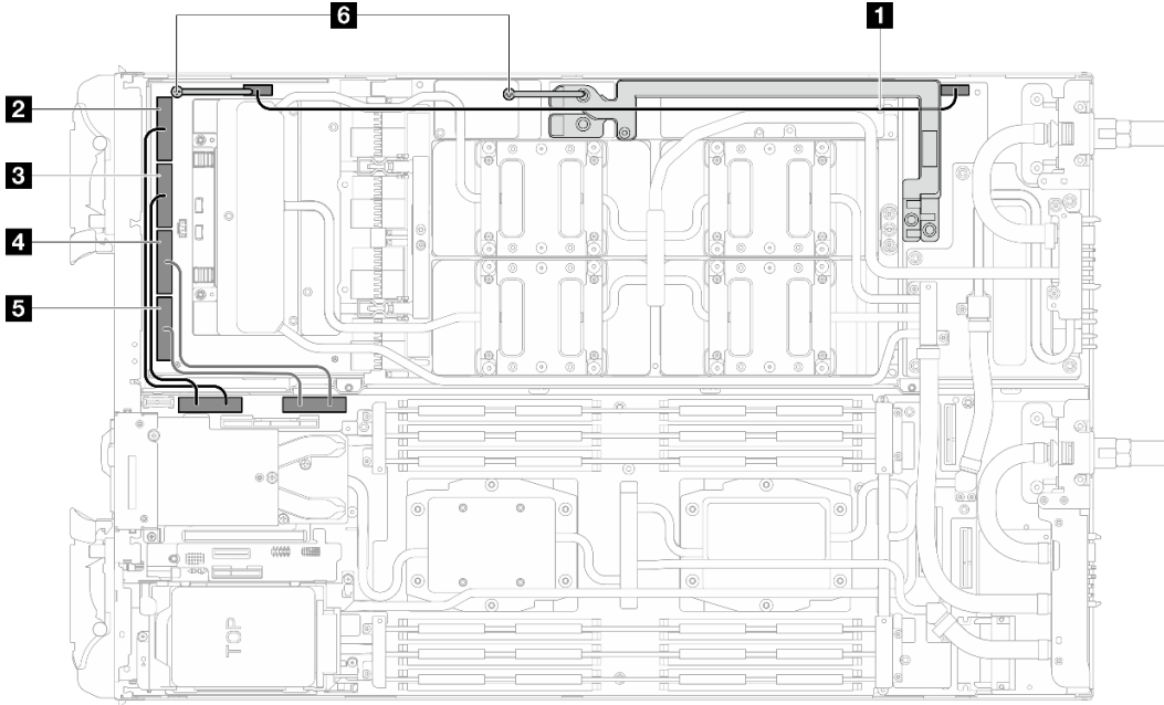
그림 452. 프로세서 1개 구성 케이블 배선
