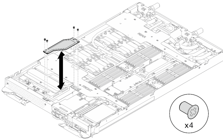
그림 7. 전면 케이블 덮개 제거
