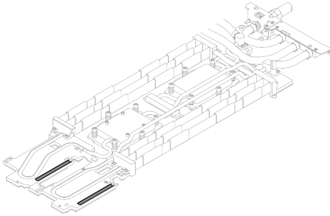
그림 45. 워터 루프 상단 갭 패드(컴퓨팅 노드 쪽)
