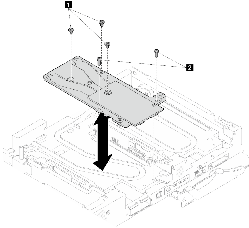
그림 183. OSFP 모듈 전도판 제거
