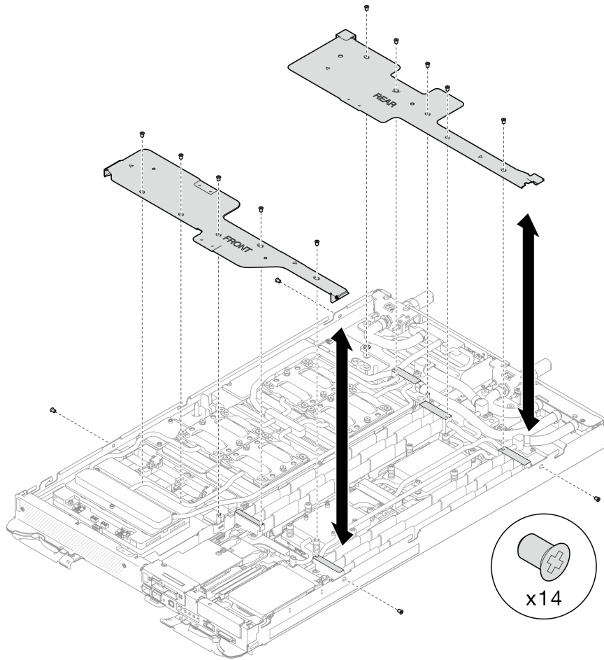
그림 8. 전면 및 후면 십자형 브레이스 제거
