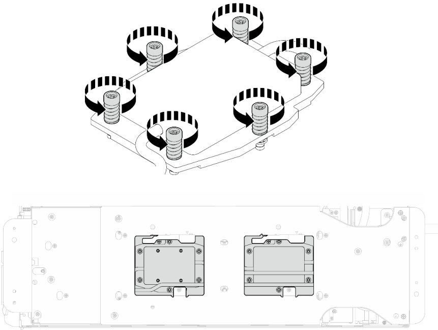
그림 188. 프로세서 냉각판 제거
