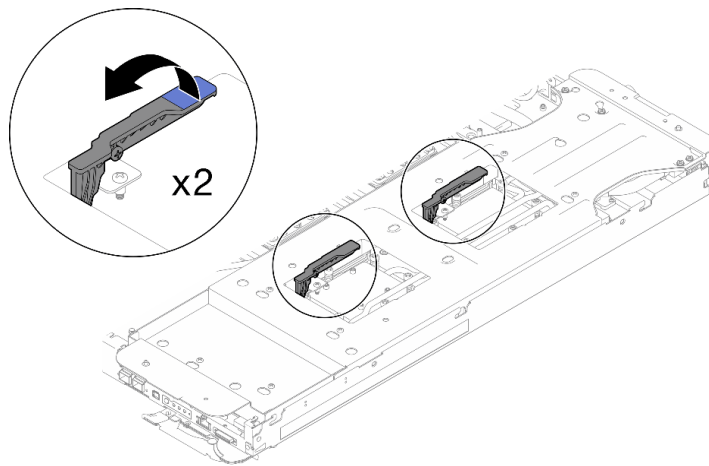
그림 250. 프로세서에서 워터 루프 분리
