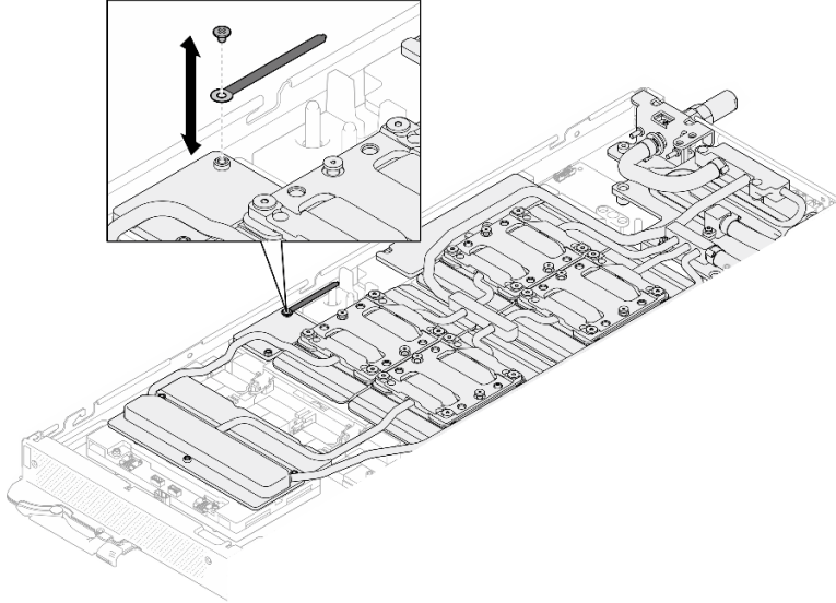
그림 12. 케이블 타이 제거
