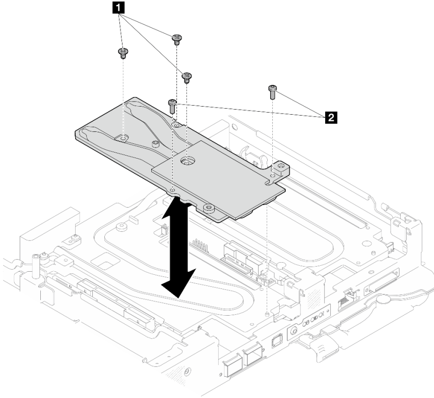
그림 28. OSFP 모듈 전도판 제거
