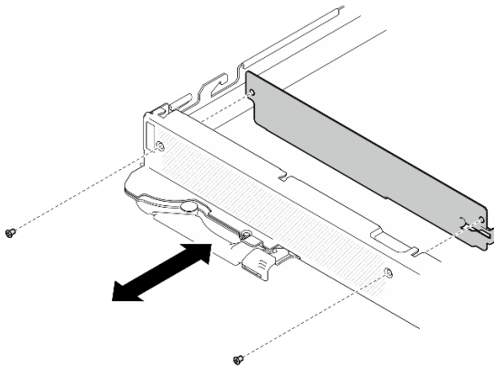
그림 449. 통풍 블록 설치
