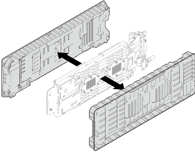
그림 41. 플라스틱 그리스 덮개 제거
