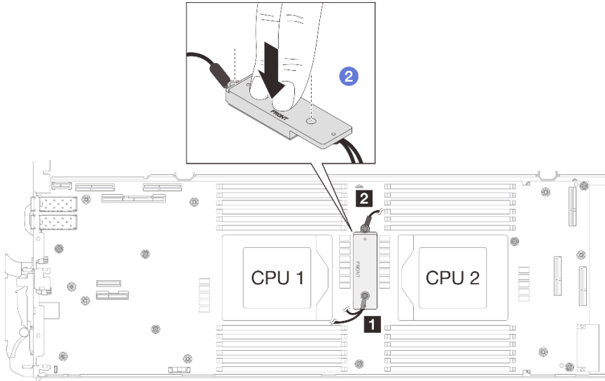
그림 281. VR 전도판 누르기
