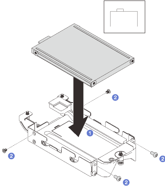
그림 134. 하단 E3.s 드라이브 설치
