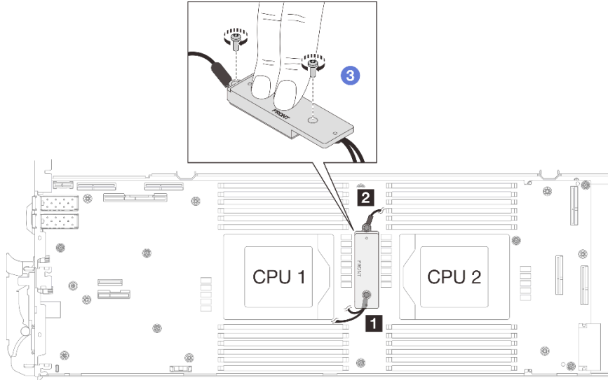
그림 75. 차폐 케이블 1/2 및 3 설치
