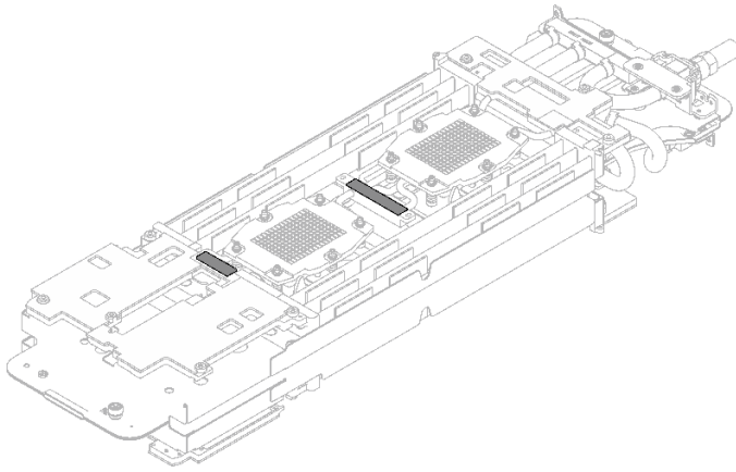
그림 43. 워터 루프 하단 퍼티 패드(컴퓨팅 노드 쪽)
