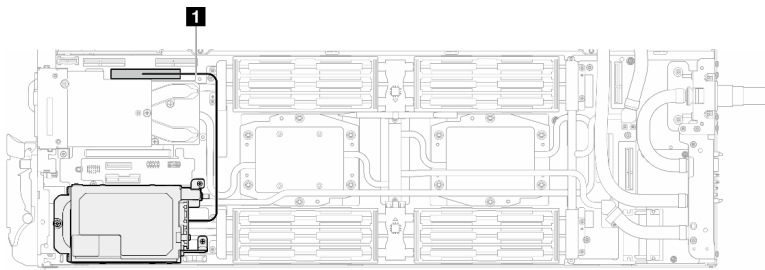
그림 167. E3.S 드라이브 케이블 연결 해제
