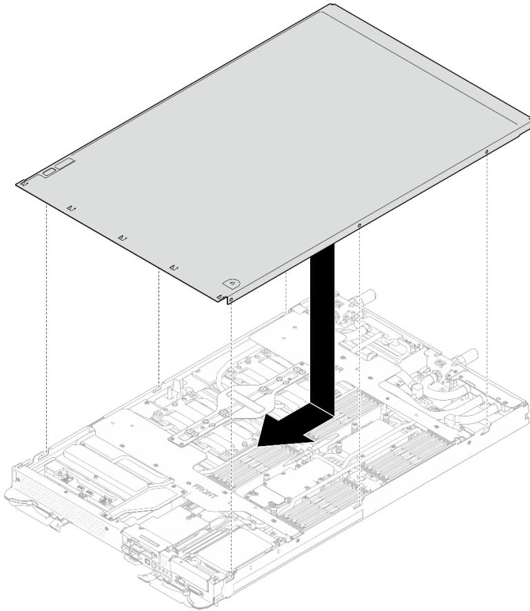
그림 6. 트레이 덮개 설치
