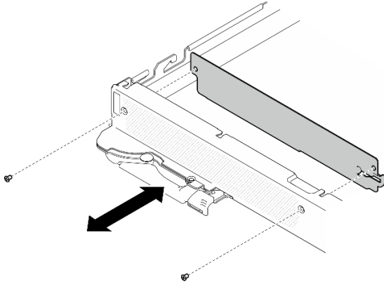
그림 448. 통풍 블록 제거
