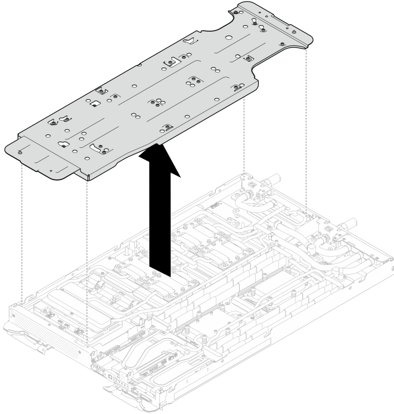
그림 61. 워터 루프 캐리어 제거(GPU 노드)
