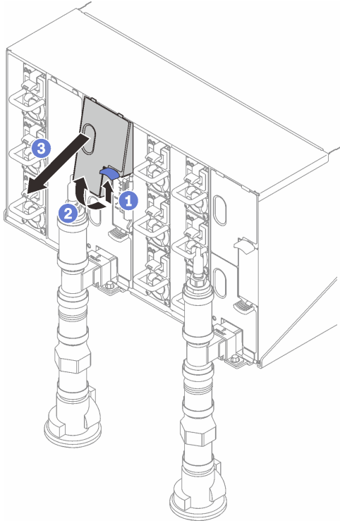
그림 466. 상단 EMC 실드 제거
