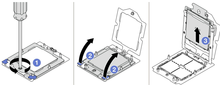
그림 222. 프로세서 제거
