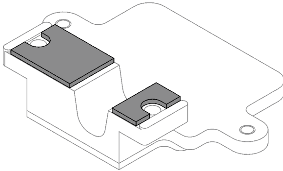
그림 147. M.2 백플레인 냉각판의 퍼티 패드(하단)
