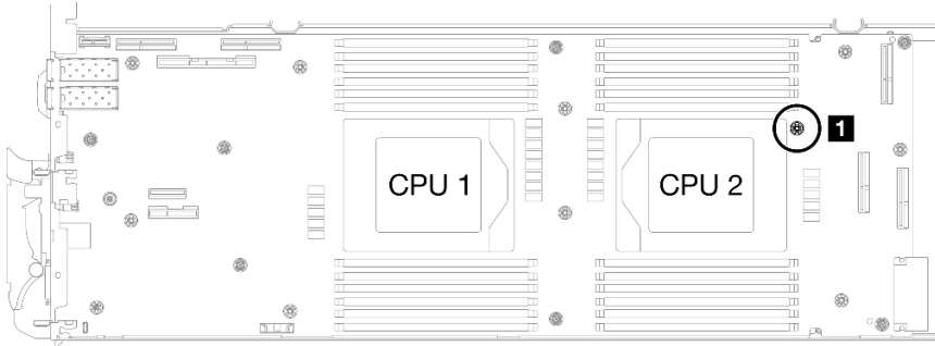
그림 283. 차폐 케이블 4의 나사 구멍 위치
