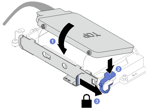
图 112. 安装上方硬盘 (7 毫米硬盘)
