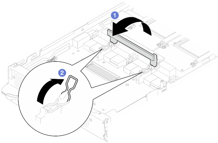
图 381. 松开载板
