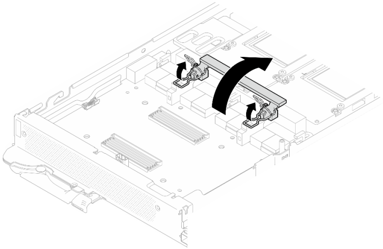
图 328. 旋转 GPU 板固定夹和手柄
