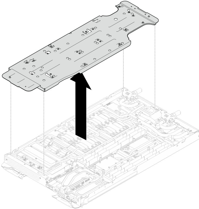
图 74. 卸下水循环模块载板 (GPU 节点)
