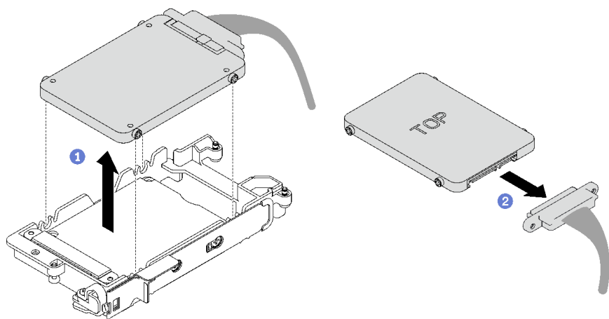
图 106. 卸下下方硬盘
