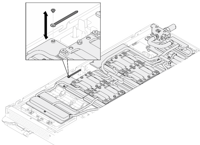
图 425. 安装线缆扎带
