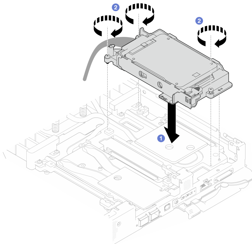
图 132. 安装 7 毫米 NVMe 硬盘仓组合件
