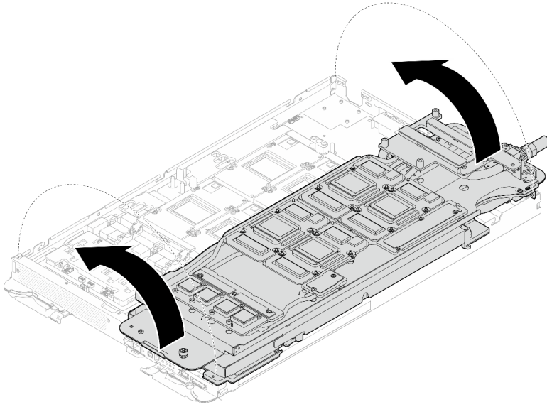
图 417. 将水循环模块展开到 GPU 节点上
