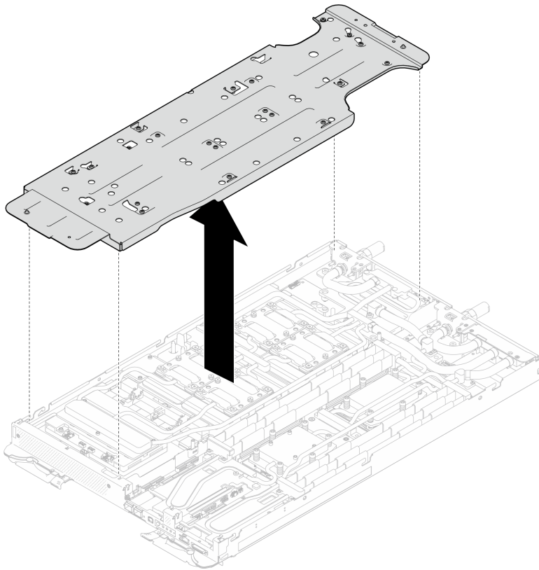
图 358. 卸下水循环模块载板 (GPU 节点)
