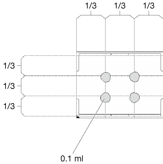
图 208. 涂抹导热油脂
