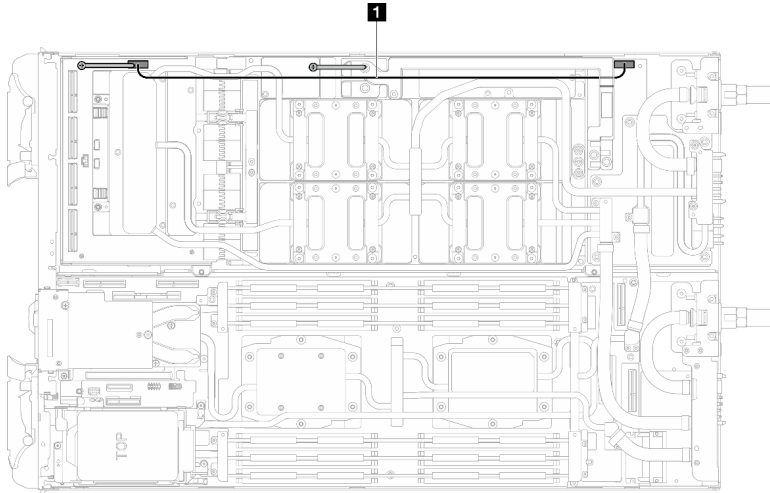
图 334. 拔下载板电源线
