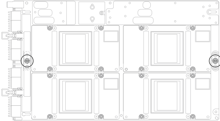
图 384. 卸下 GPU 板组合件 T15 螺钉
