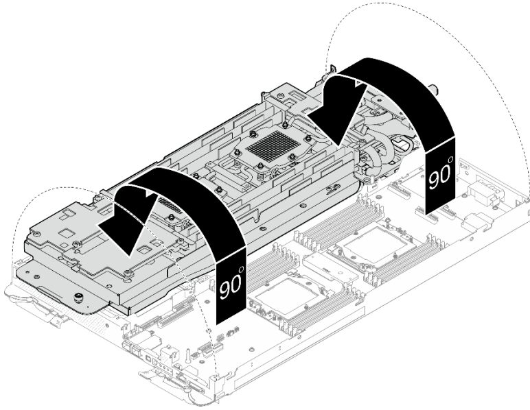
图 264. 折叠水循环模块
