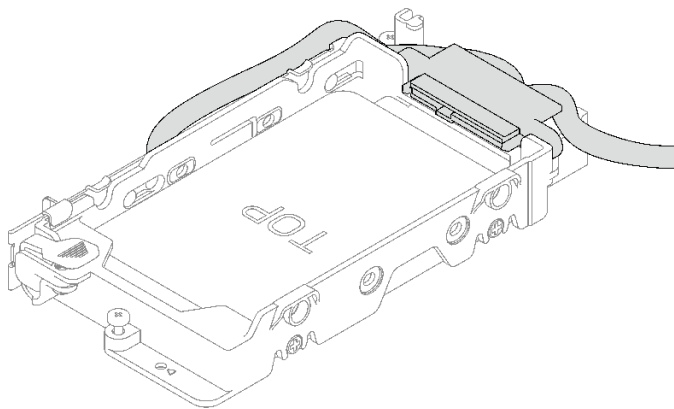
图 109. 固定未插入的线缆插头
