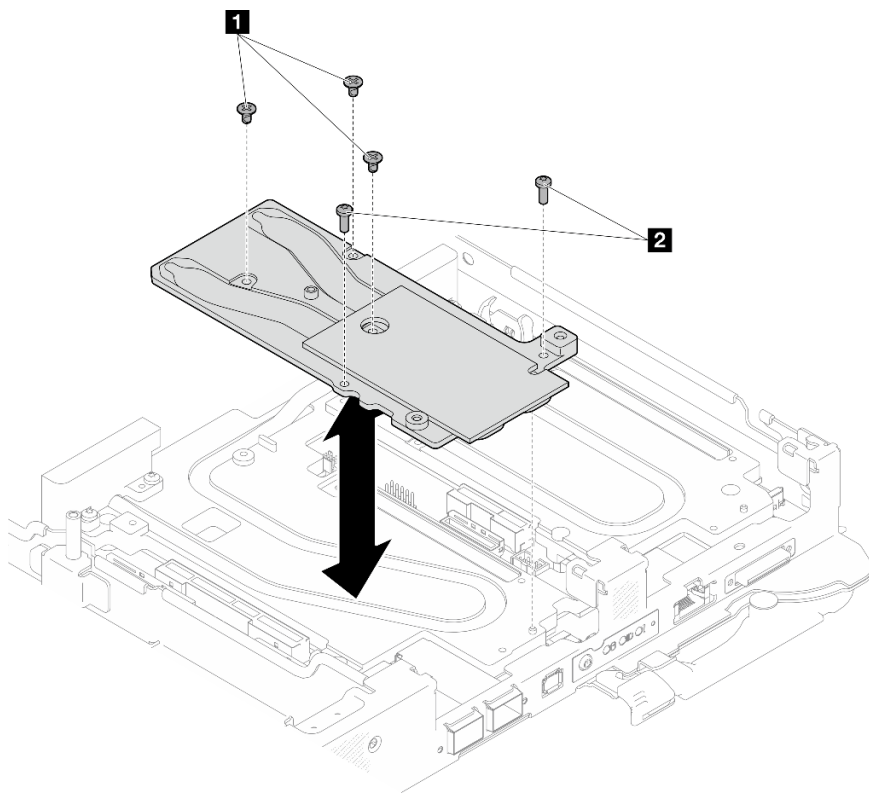
图 225. 卸下 OSFP 模块导电板
