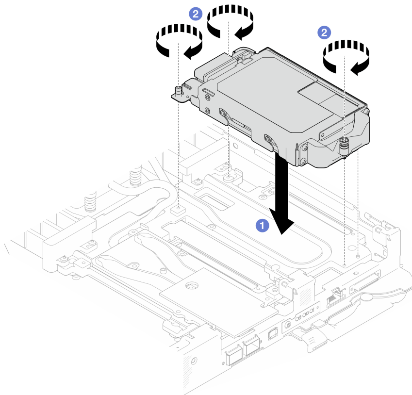
图 153. 安装 E3.S 硬盘仓组合件
