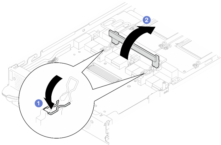
图 391. 将载板固定到 GPU 板上
