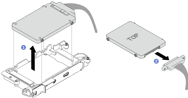
图 104. 卸下一个 7 毫米硬盘
