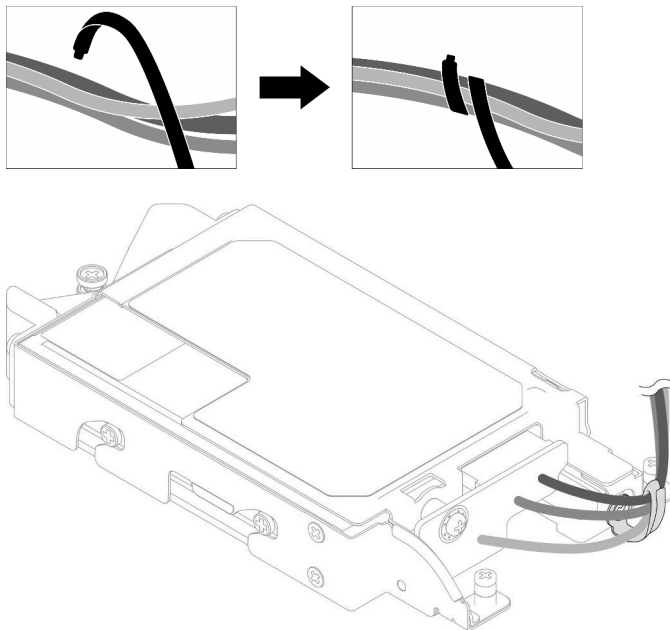
图 150. 用线缆扎带捆扎线缆
