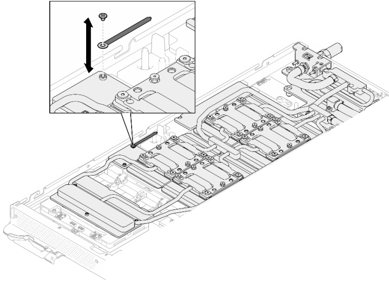
图 395. 取下线缆扎带
