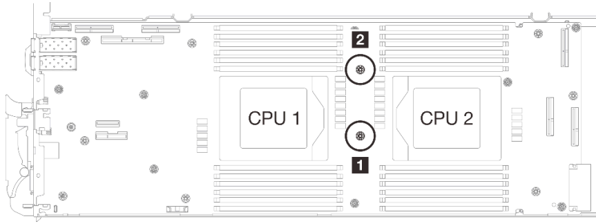
图 84. 屏蔽线缆 1/2 和 3 的螺钉孔的位置
