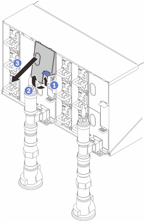
图 479. 卸下上方 EMC 保护罩
