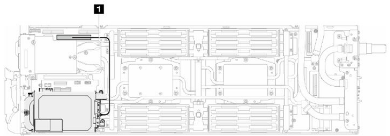
图 194. 连接 E3.S 硬盘线缆
