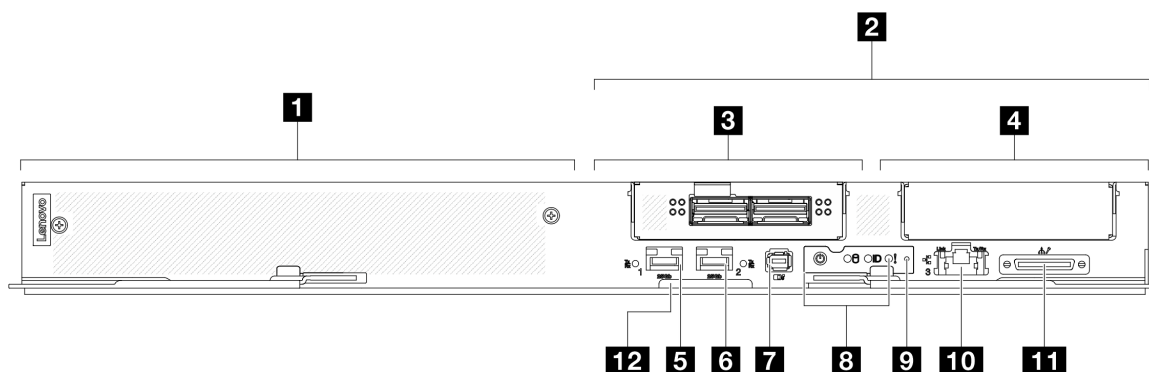
图 2. SD665-N V3 托盘
