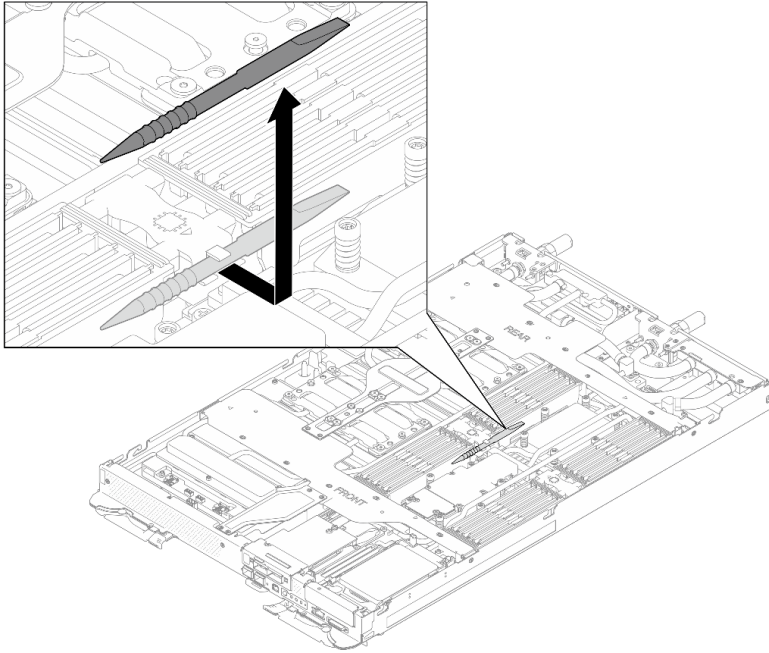
图 173. 卸下内存条工具
