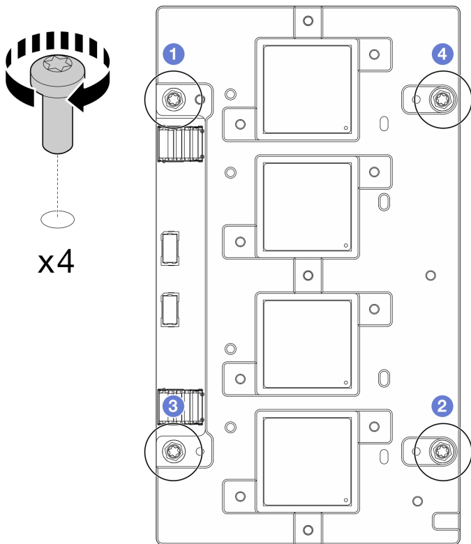
图 446. 安装网卡螺钉
