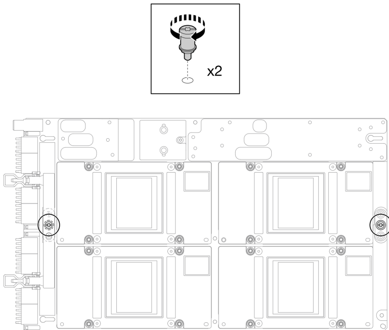
图 389. 将 T15 螺钉安装到 GPU 板组合件上
