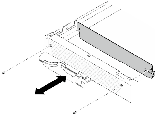
图 461. 卸下通风块
