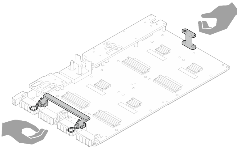
图 373. 从包装盒中取出 GPU 板
