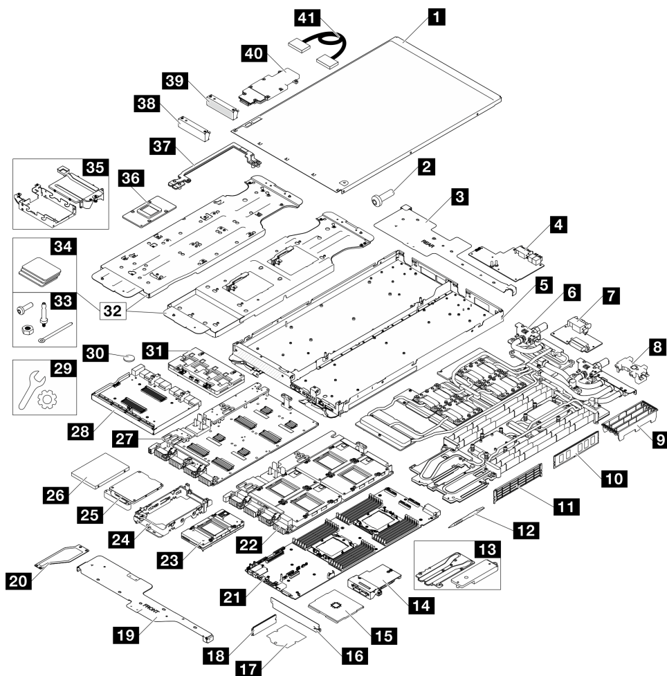
图 11. SD665-N V3 部件列表
