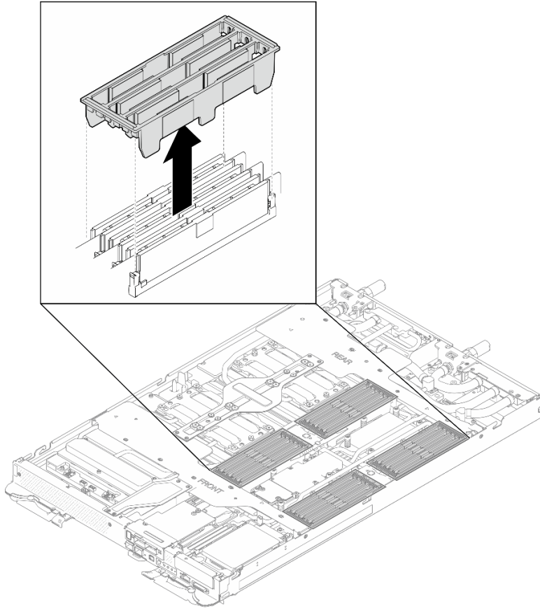
图 174. 卸下 DIMM 外盖
