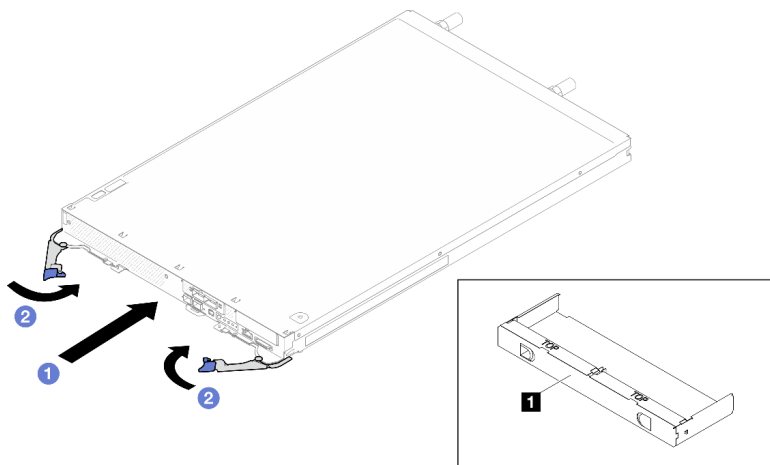
图 17. 安装托盘
