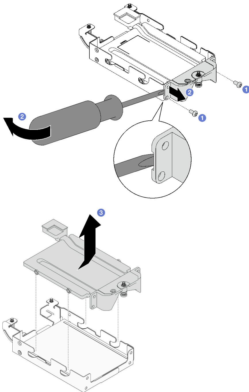
图 141. 卸下导电板
