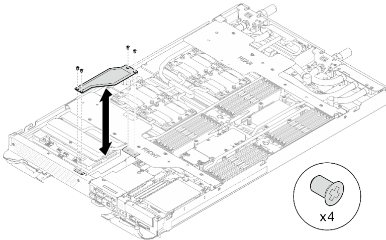
图 20. 卸下正面线缆外盖
