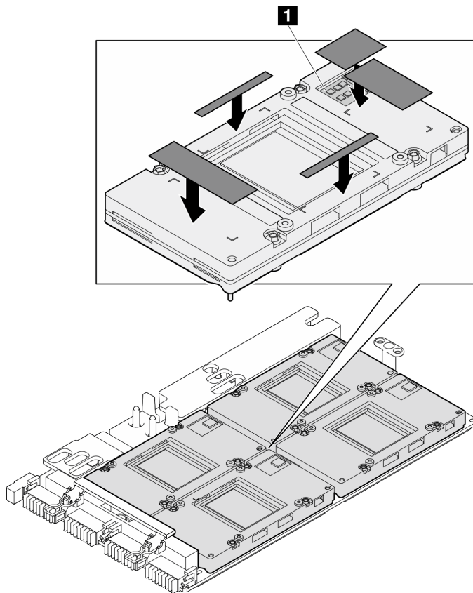
图 61. 更换 GPU 油灰垫
