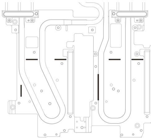
图 130. 水循环模块上的间隙垫对齐标记
