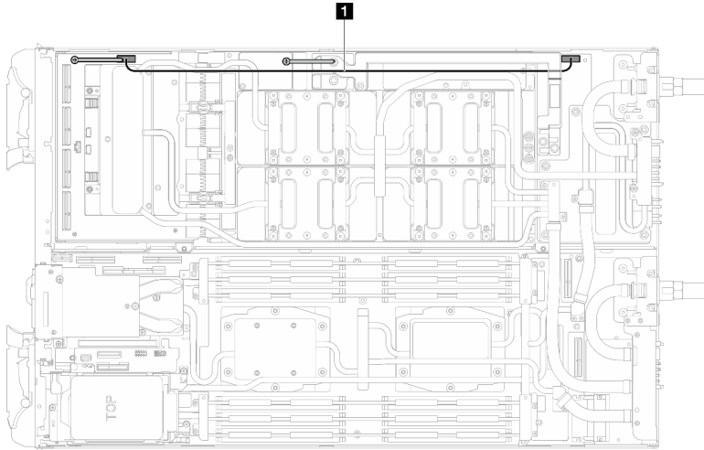
图 332. 连接载板电源线
