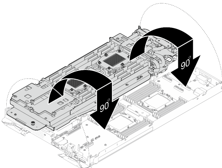
图 244. 安装水循环模块
