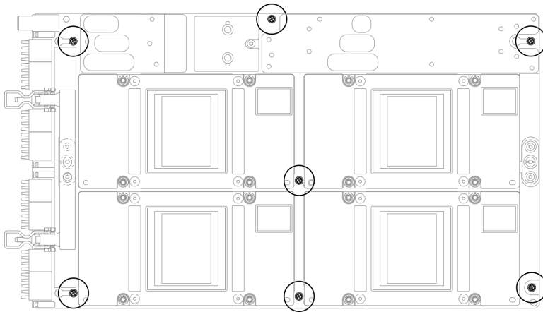
图 383. 卸下 GPU 板组合件 M3 螺钉
