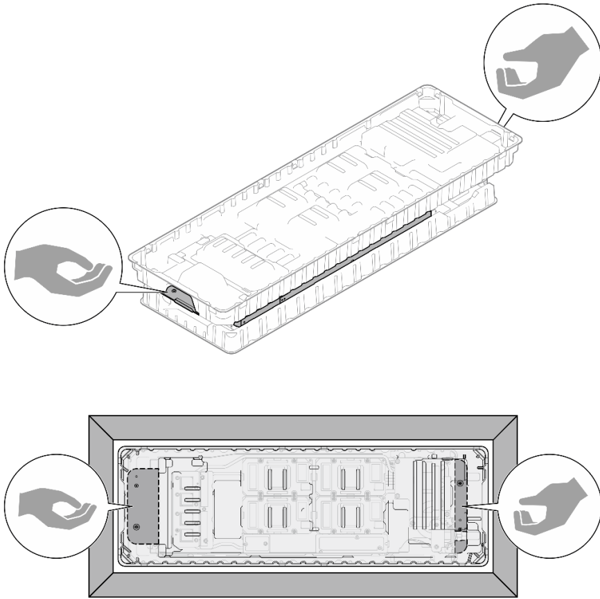
图 53. 从包装盒中取出水循环模块时的操作点
