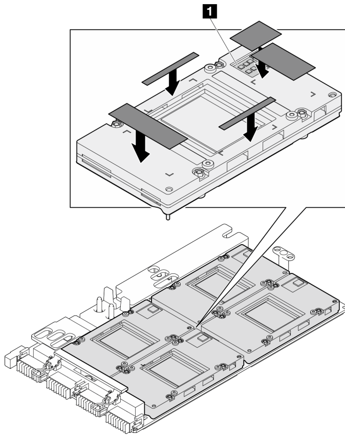
图 416. 更换 GPU 油灰垫
