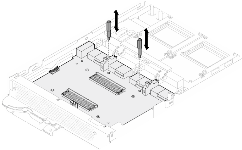
图 392. 安装载板支脚
