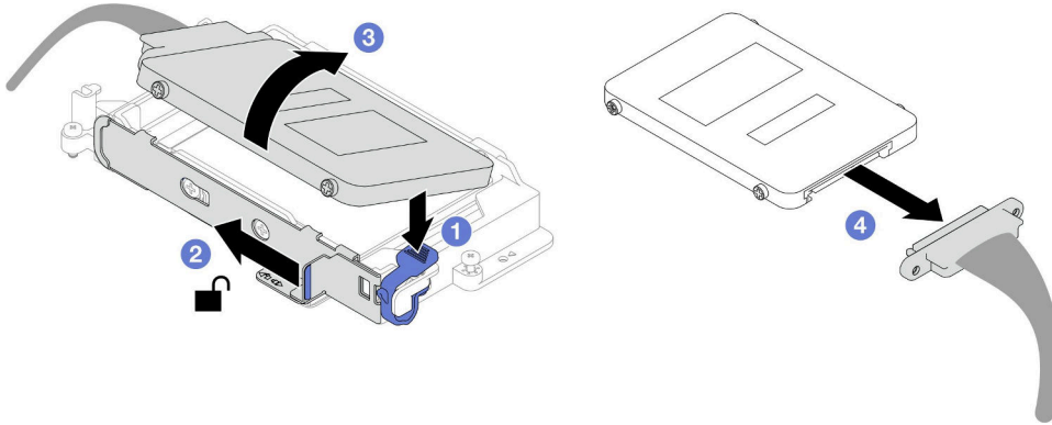
图 123. 卸下上方硬盘（7 毫米 NVMe）
