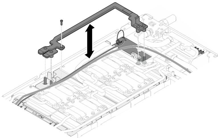
图 324. 安装汇流条
