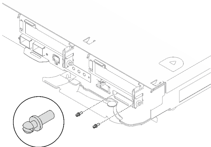
图 307. 安装 KVM 螺钉
