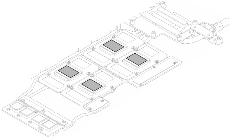
图 37. 清除所有 GPU 上的 PCM
