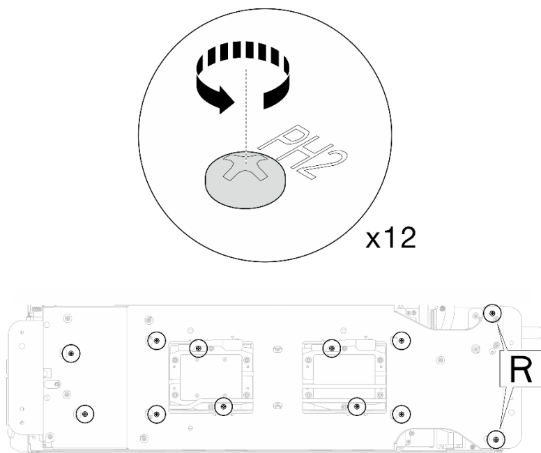
图 64. 拧松水循环模块载板的螺钉
