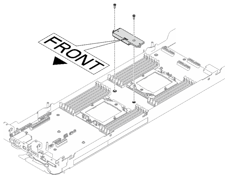
图 89. 卸下 VR 导电板
