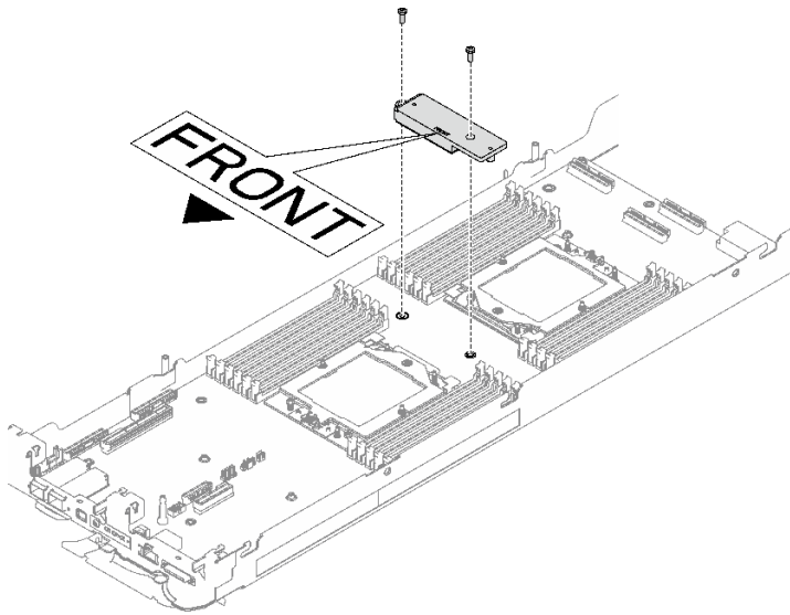
图 91. 卸下 VR 导电板
