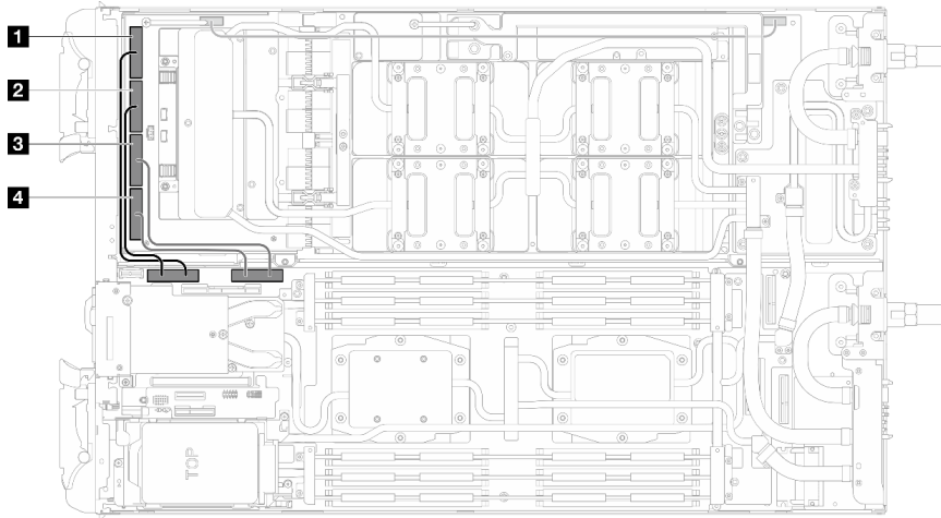
图 191. 单处理器配置 — 将所有 MCIO 线缆连接到载板
