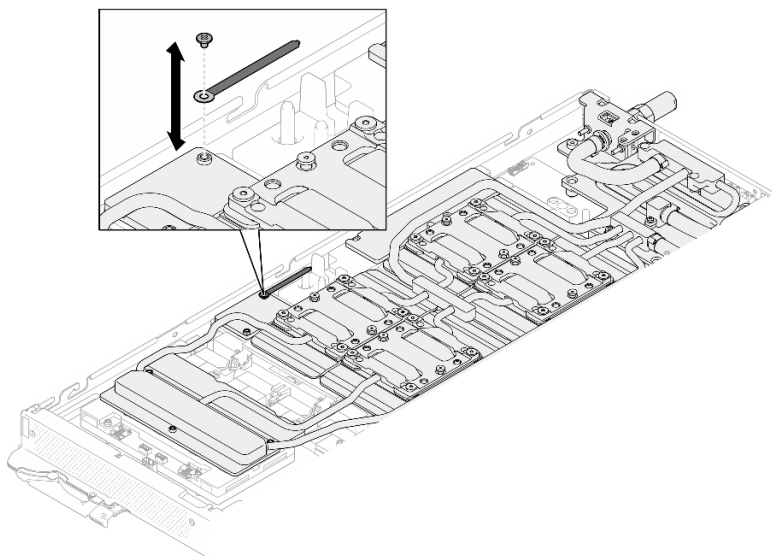
图 429. 取下线缆扎带
