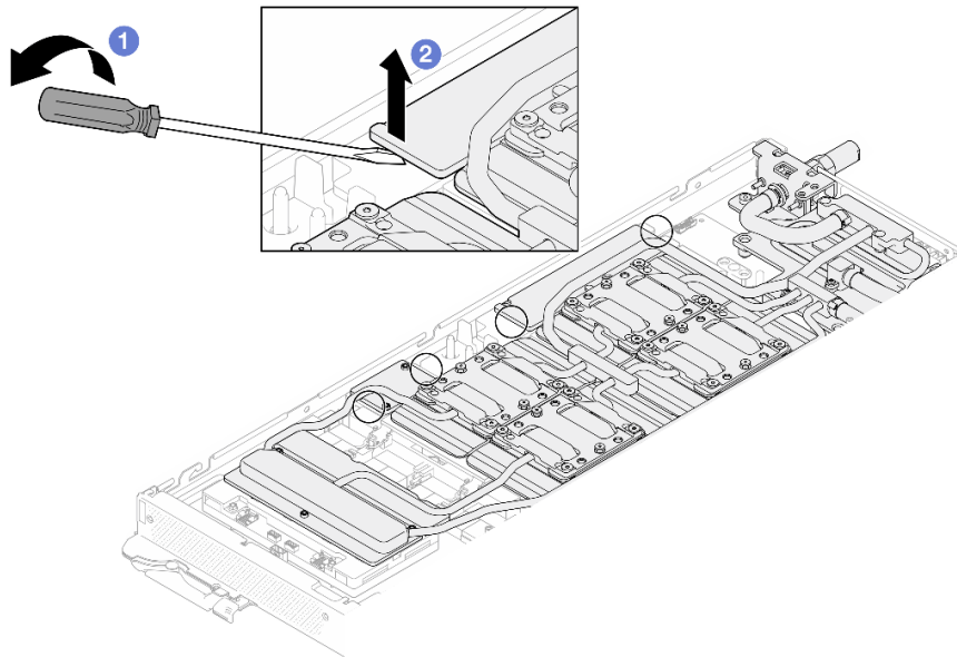
图 31. 从 GPU 板上松开正面和背面 MISC 导电板
