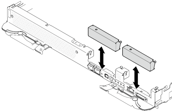
图 113. 安装空挡板填充件
