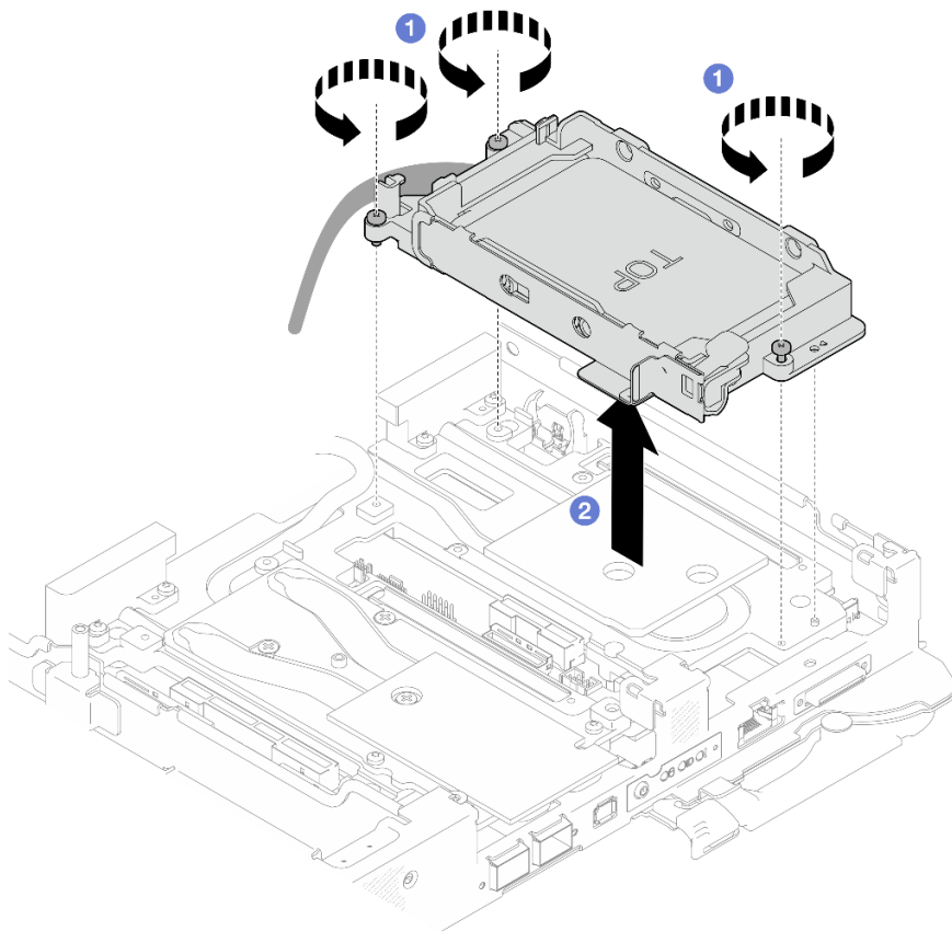
图 101. 卸下单 7 毫米硬盘仓组合件
