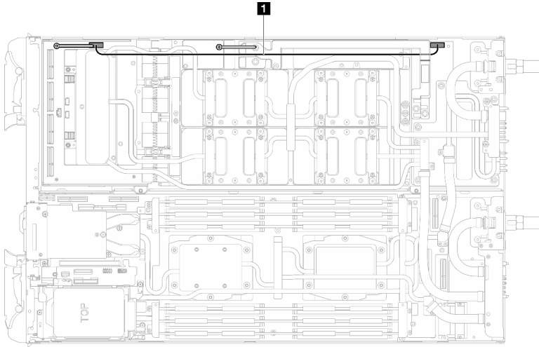
图 426. 连接载板电源线
