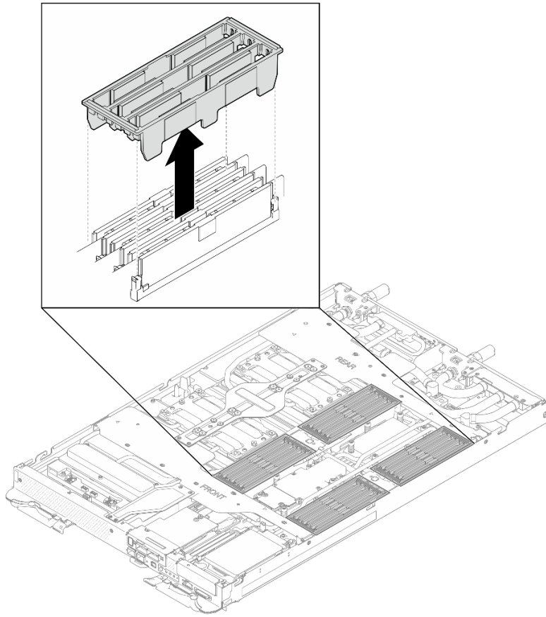
图 167. 卸下 DIMM 外盖
