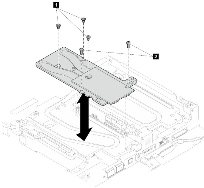
图 71. 安装 OSFP 模块导电板
