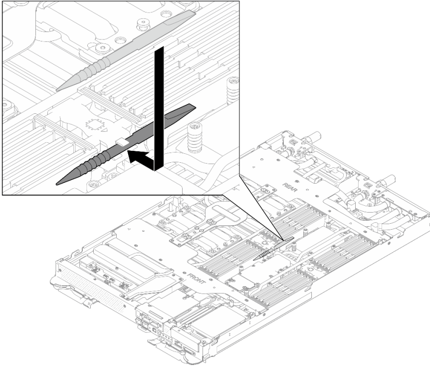
图 178. 内存条工具
