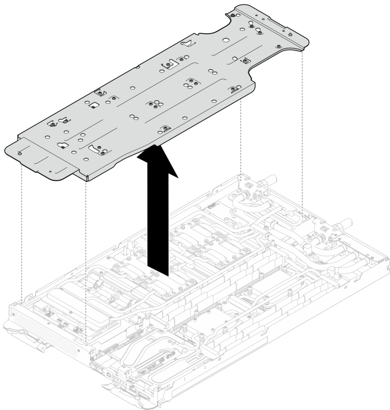
图 419. 卸下水循环模块载板 (GPU 节点)
