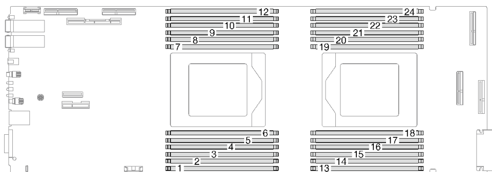
图 172. 内存条插槽位置
