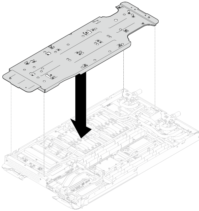
图 438. 安装水循环模块载板 (GPU 节点)
