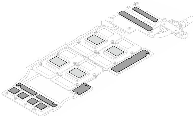
图 448. 更换水循环模块油灰垫 (GPU 节点)
