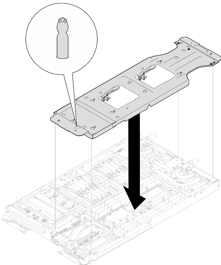
图 261. 安装水循环模块载板（计算节点）
