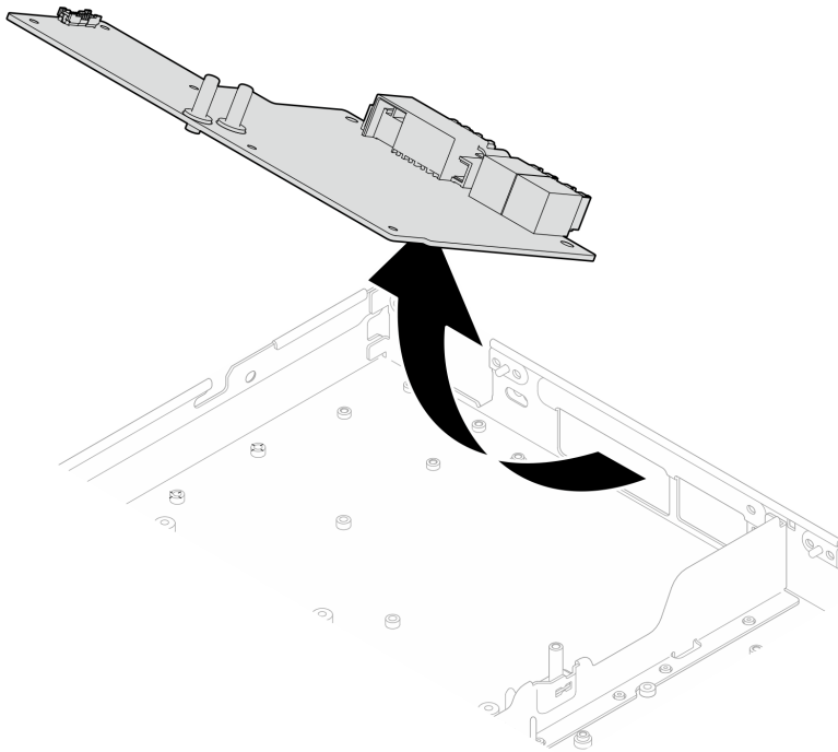
图 410. 卸下 GPU 配电板
