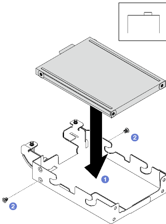
图 143. 安装顶部 E3.s 硬盘
