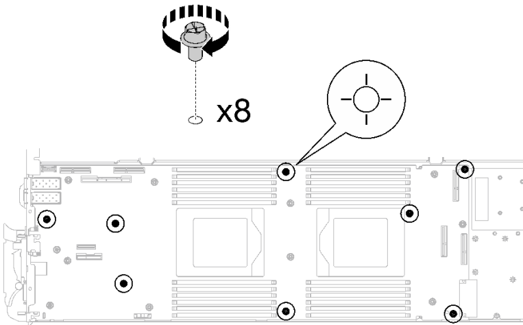
图 285. 卸下主板螺钉
