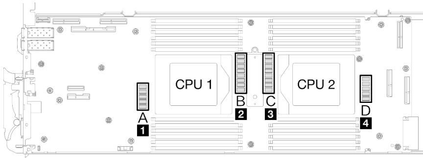
图 301. 主板上的电感器位置
