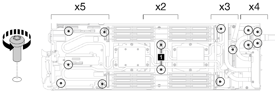
图 44. 卸下水循环模块螺钉
