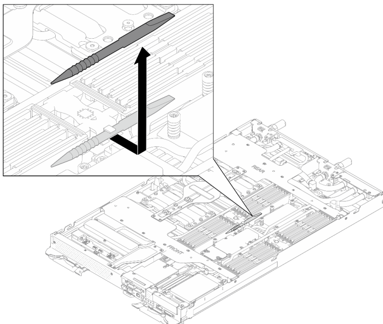
图 166. 卸下内存条工具
