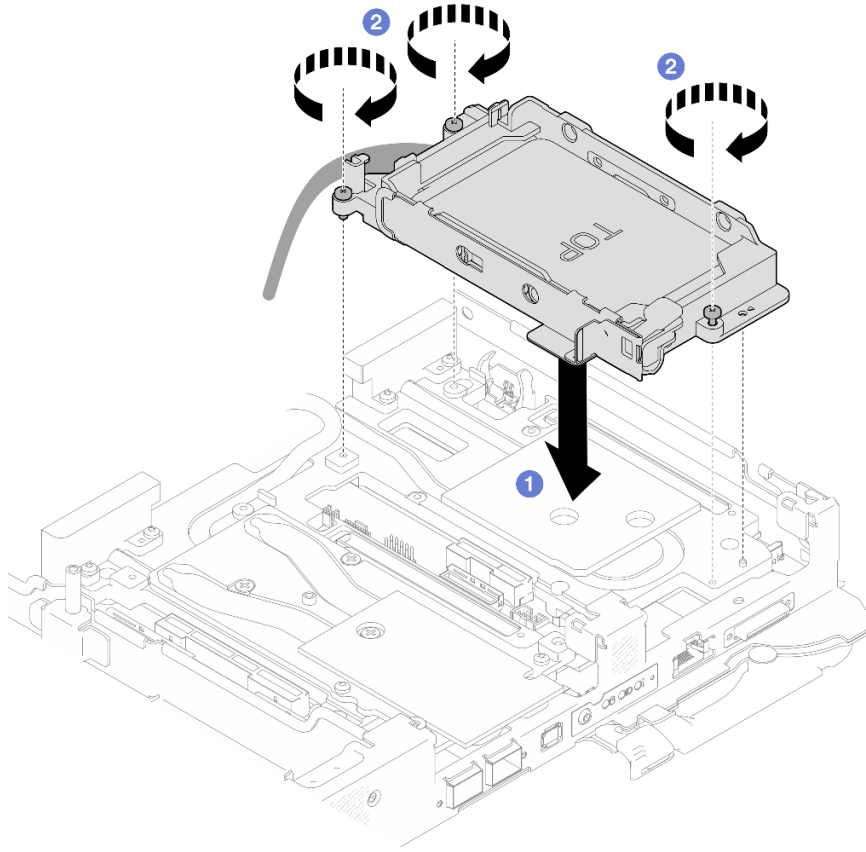
图 117. 安装单 7 毫米硬盘仓组合件
