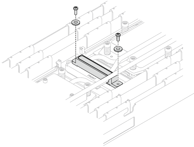
图 217. VR 冷却板螺钉以及垫圈
