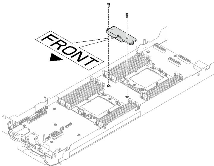
图 82. 卸下 VR 导电板
