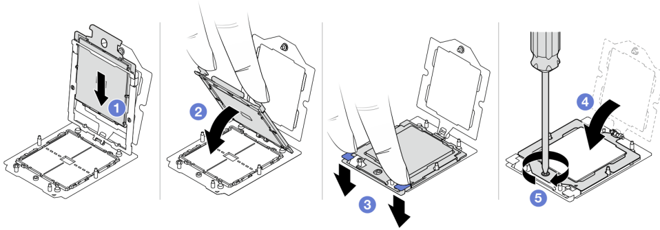
图 237. 安装处理器
