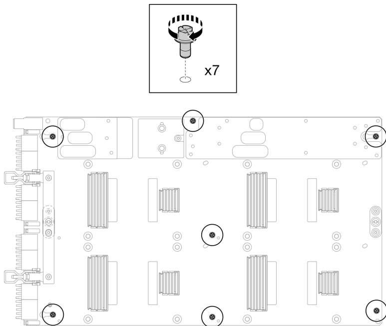
图 375. 将 M3 螺钉安装到 GPU 板上
