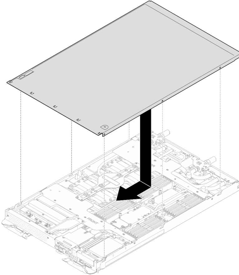
图 19. 安装托盘外盖
