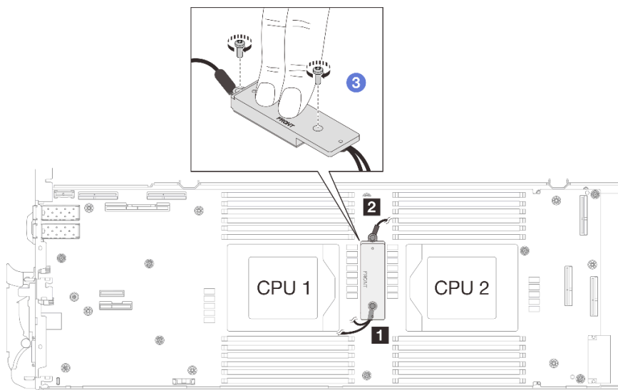
图 312. 连接屏蔽线缆 1/2 和 3
