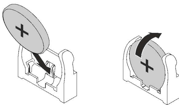
图 95. 安装 CMOS 电池
