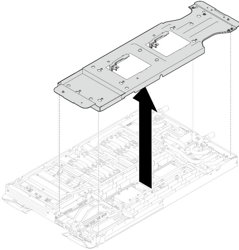
图 246. 卸下水循环模块载板 (计算节点)
