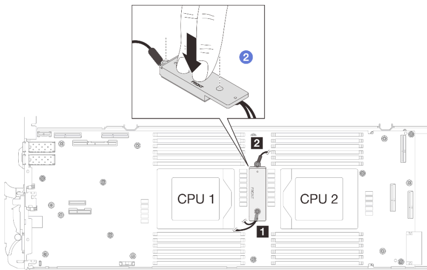
图 311. 按压 VR 导电板
