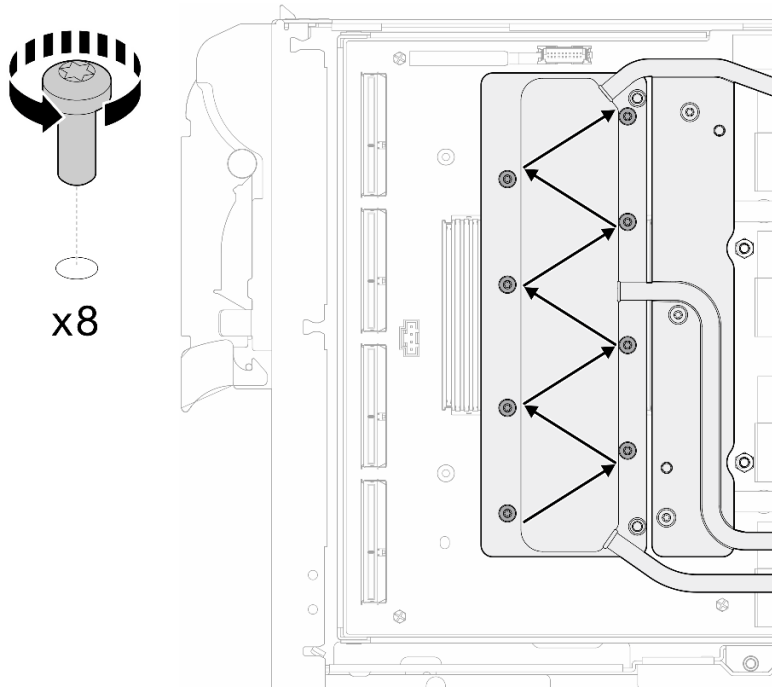
图 399. 卸下网卡螺钉
