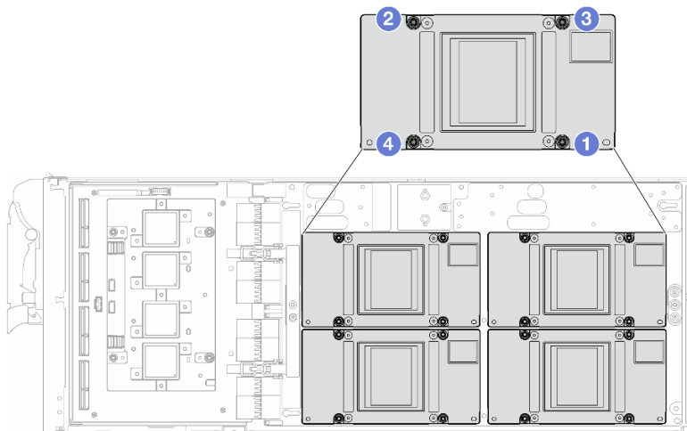
图 352. GPU 螺钉拧紧顺序
