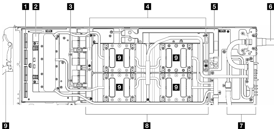
图 4. GPU 节点俯视图
