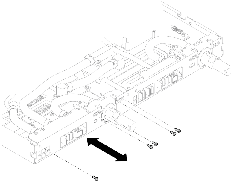
图 219. 安装快接件螺钉 (计算节点)
