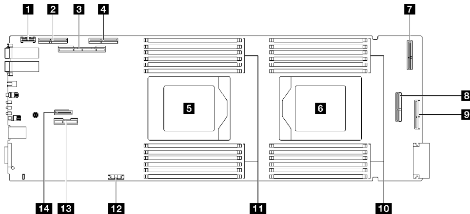
图 8. 计算节点主板上的内部接口
