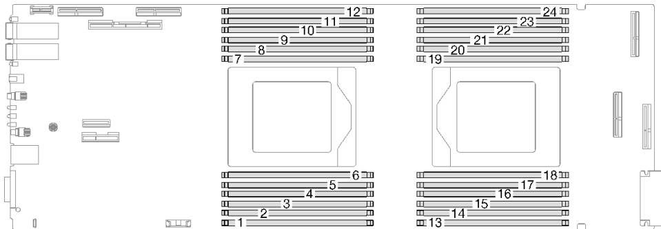
图 7. 计算节点主板上的 DIMM 插槽编号
