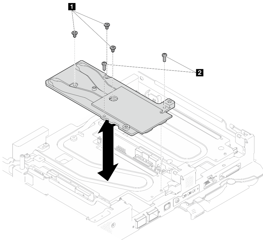
图 196. 卸下 OSFP 模块导电板
