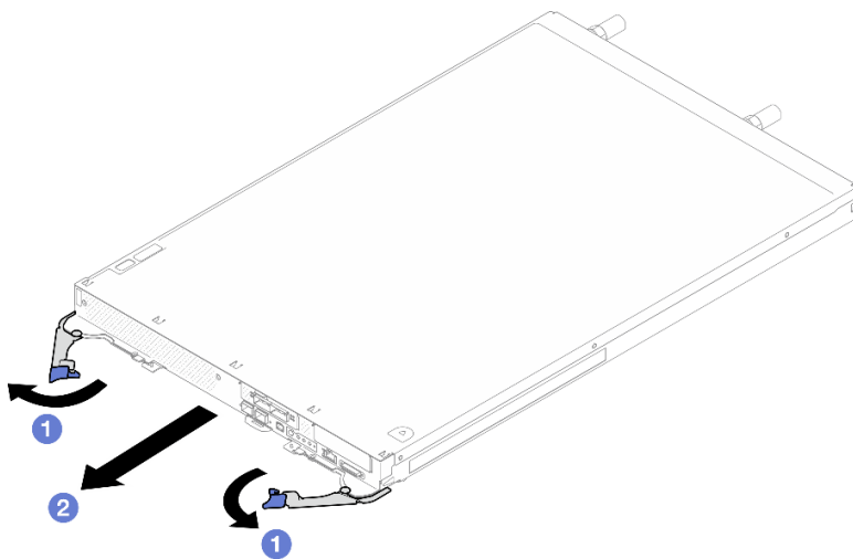
图 16. 卸下托盘
