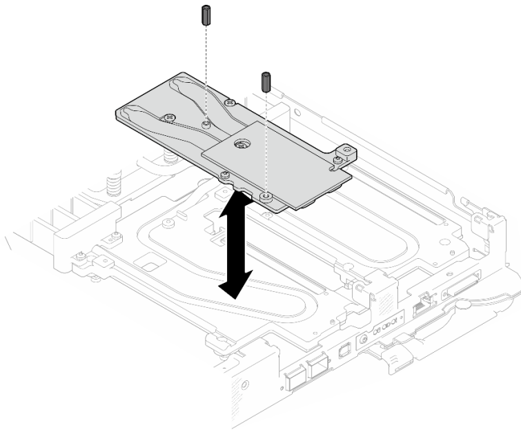
图 40. 卸下 OSFP 模块导电板六角螺钉
