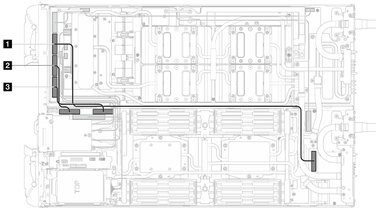
图 192. 双处理器配置 — 将 MCIO 2、MCIO 3 和 MCIO 4 线缆连接到 GPU 节点
