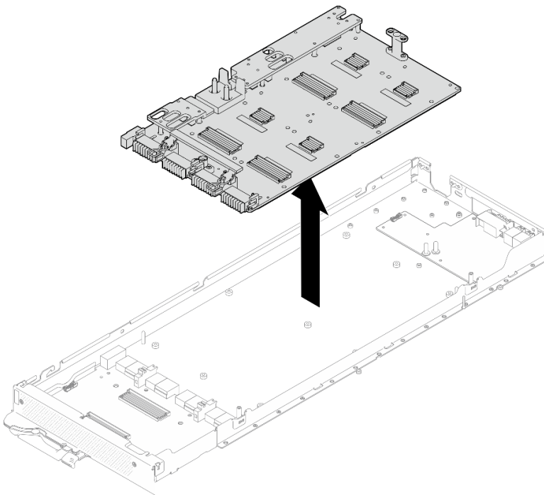
图 371. 卸下 GPU 板
