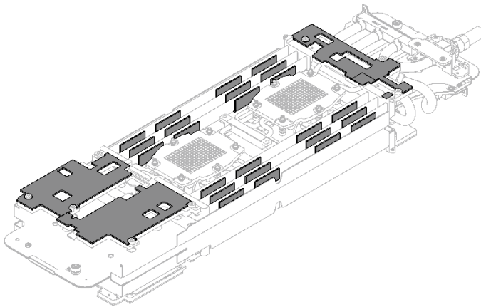
图 240. 水循环模块间隙垫（底面）
