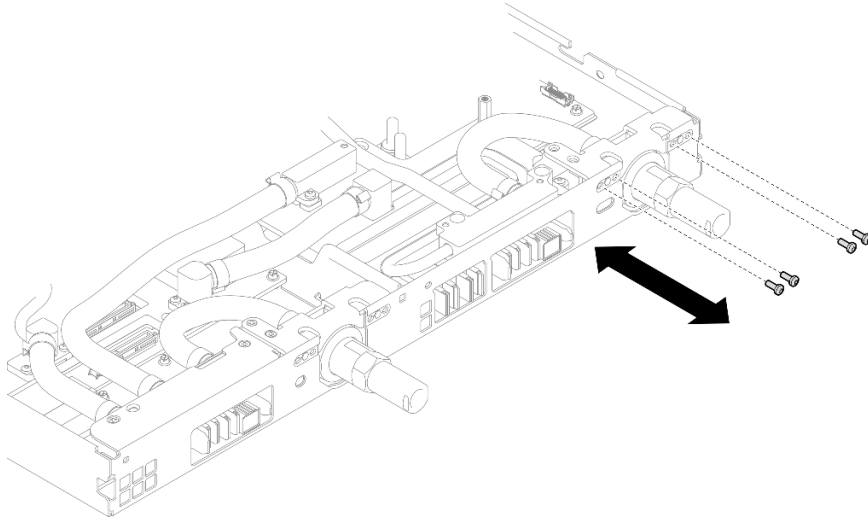
图 432. 卸下快接件螺钉 (GPU 节点)
