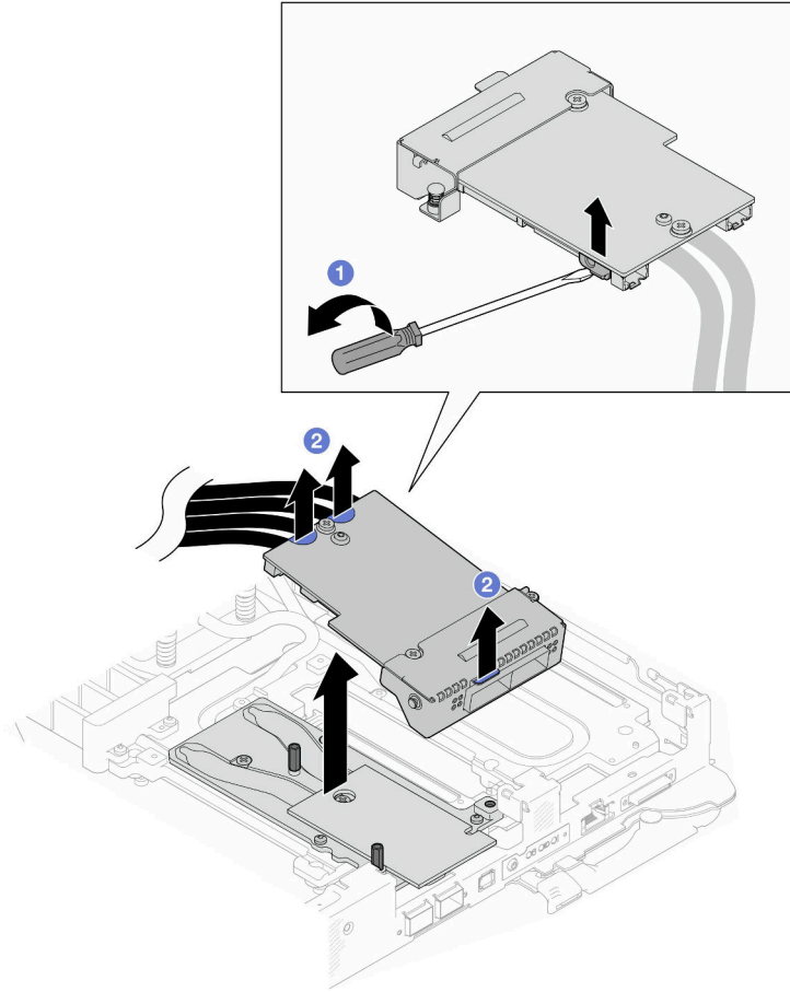
图 185. 卸下 OSFP 模块
