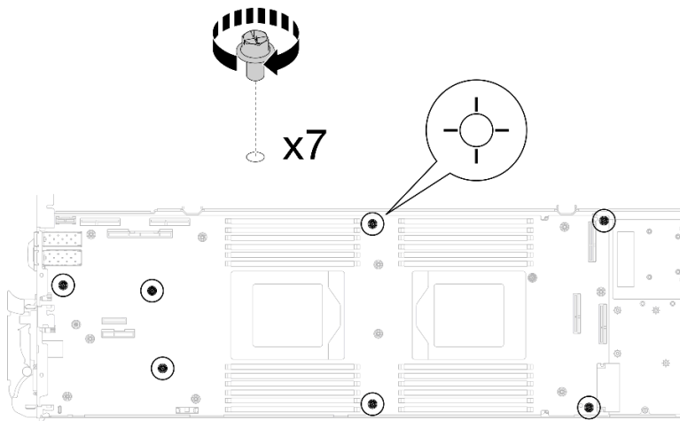
图 316. 安装主板螺钉
