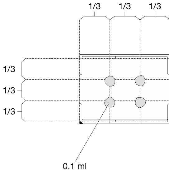
图 238. 涂抹导热油脂
