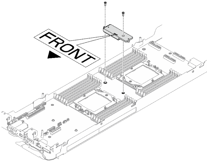
图 284. 卸下 VR 导电板
