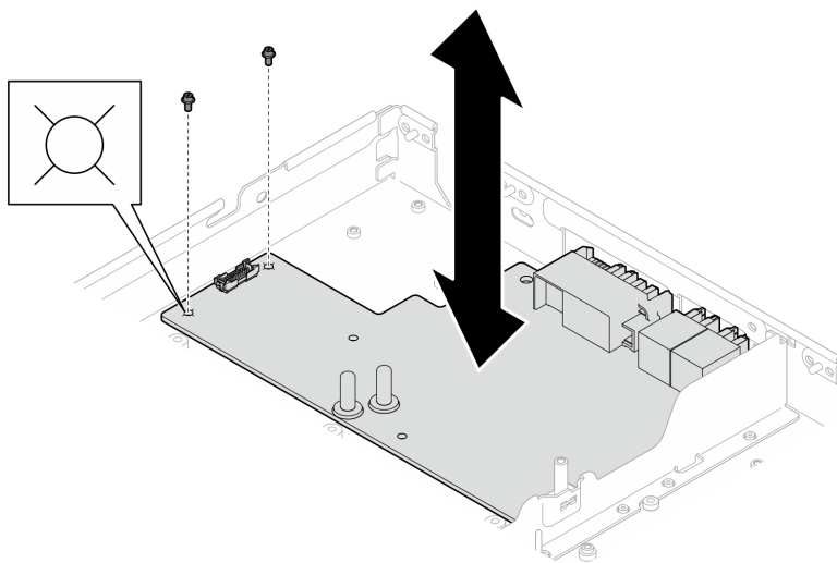
图 413. 安装 GPU 配电板螺钉
