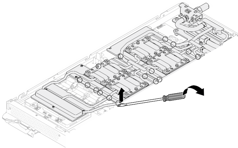
图 33. 从 GPU 上松开 GPU 冷却板
