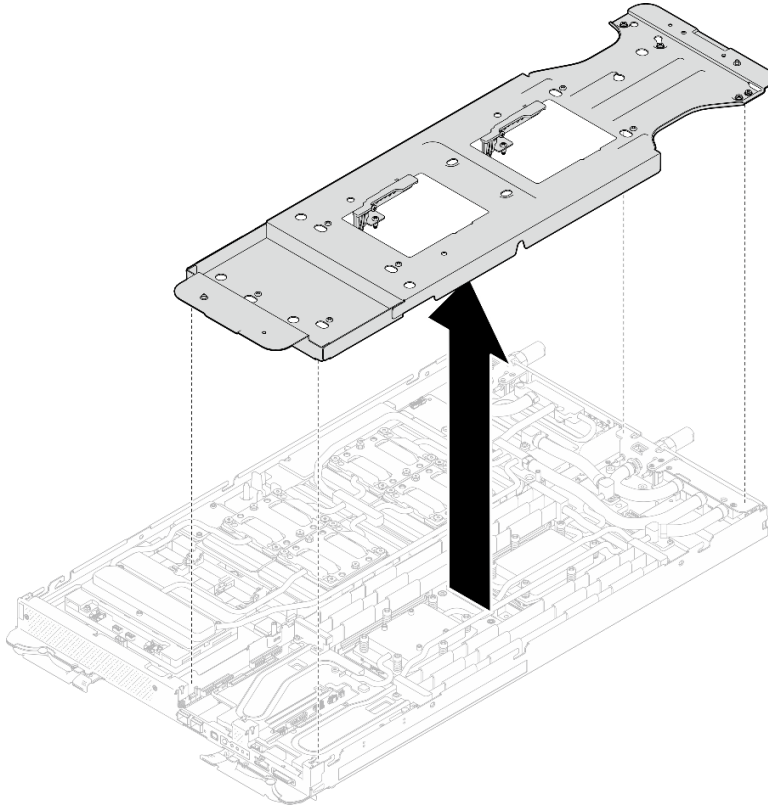
图 215. 卸下水循环模块载板（计算节点）
