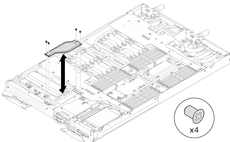
图 23. 安装正面线缆外盖
