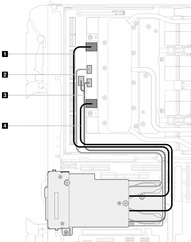
图 427. 从网卡上拔下 OSFP 模块线缆
