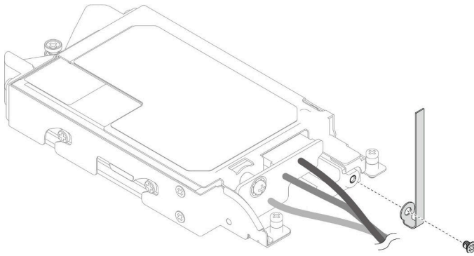
图 149. 安装线缆扎带
