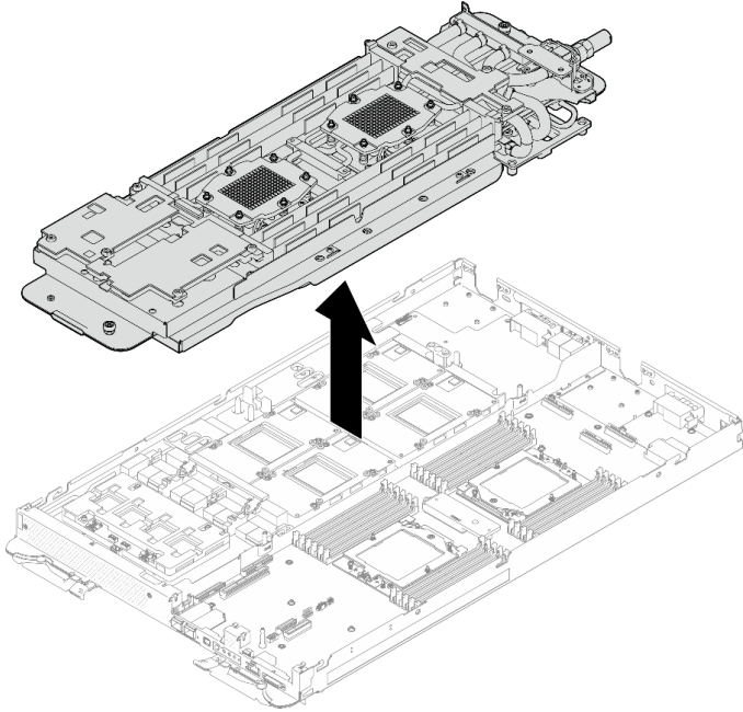
图 52. 卸下水循环模块
