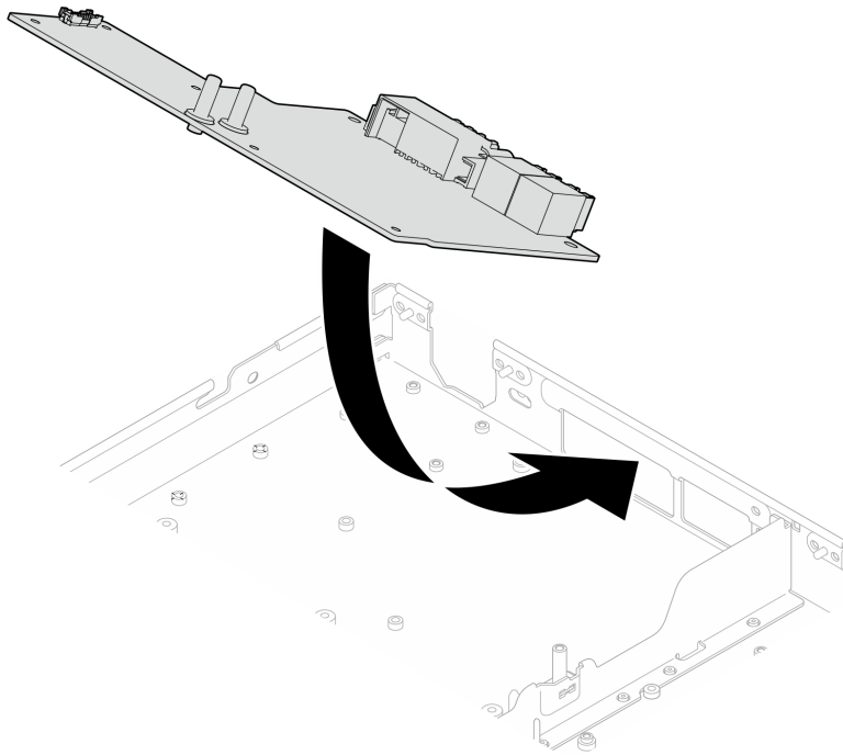
图 412. 安装 GPU 配电板
