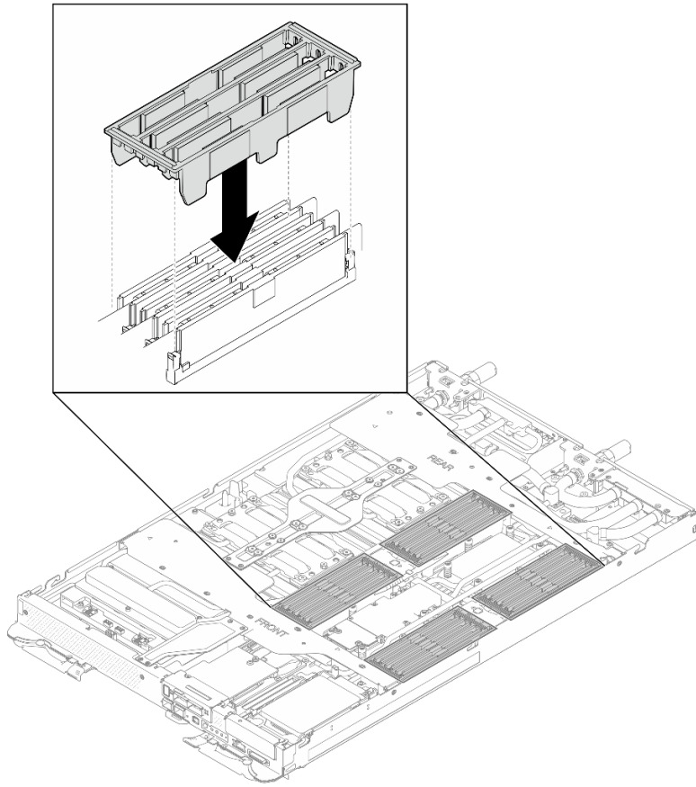
图 177. 安装 DIMM 外盖
