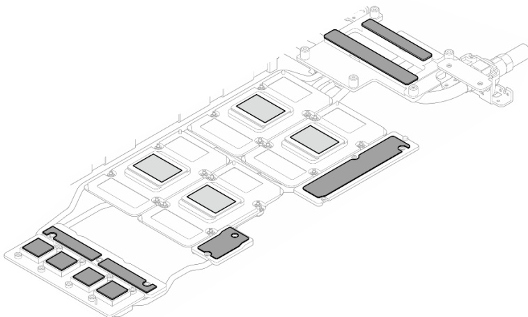
图 415. 更换水循环模块油灰垫 (GPU 节点)
