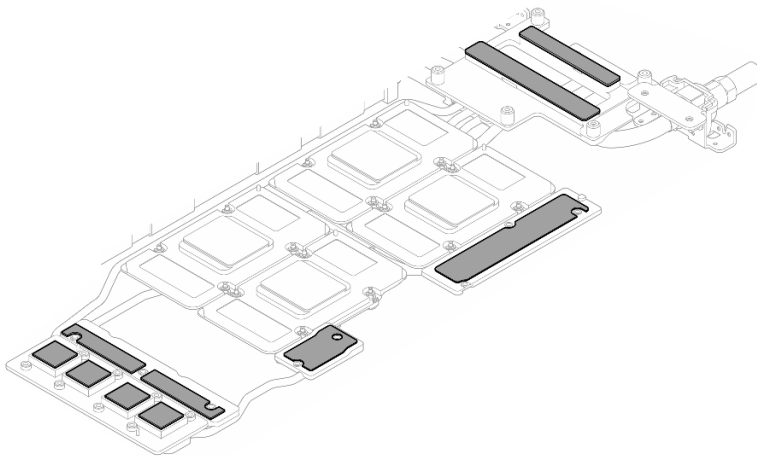
图 348. 清除水循环模块上的油灰垫
