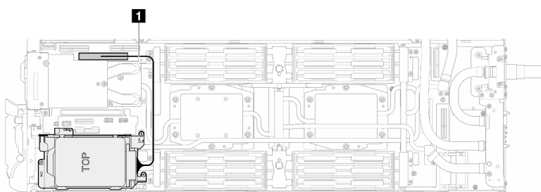
图 133. 连接硬盘仓线缆
