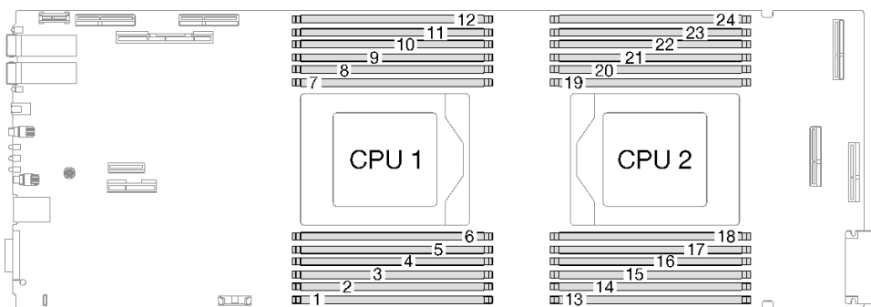
图 14. 内存条和处理器布局
