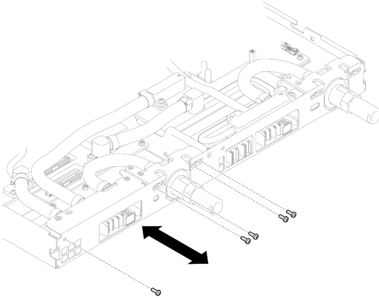
图 226. 卸下快接件螺钉（计算节点）
