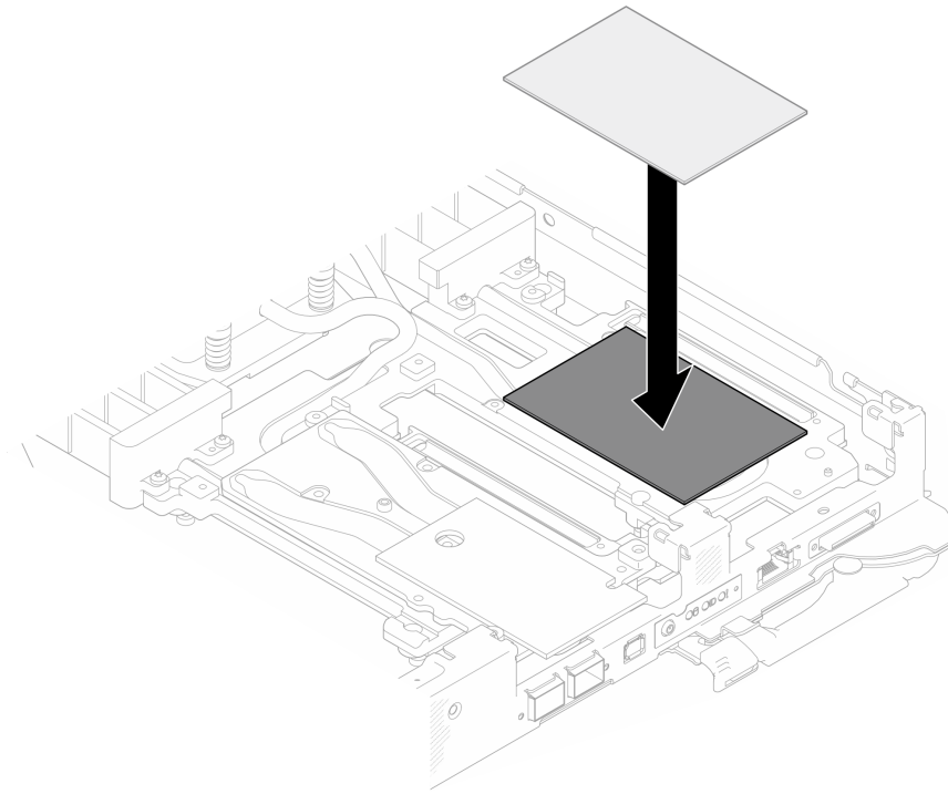
图 152. 更换间隙垫
