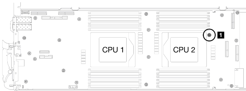
图 313. 屏蔽线缆 4 的螺钉孔的位置
