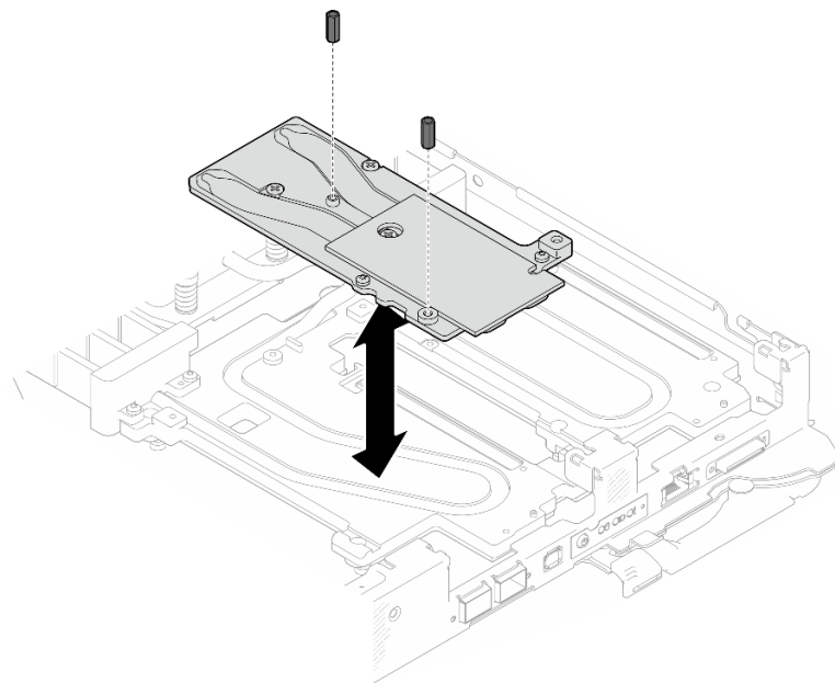
图 254. 卸下 OSFP 模块导电板六角螺钉
