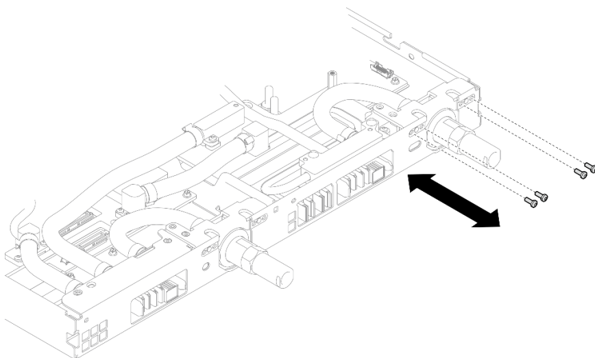
图 338. 卸下快接件螺钉 (GPU 节点)
