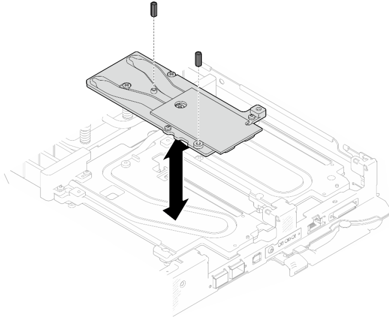
图 72. 安装 OSFP 模块导电板六角螺钉
