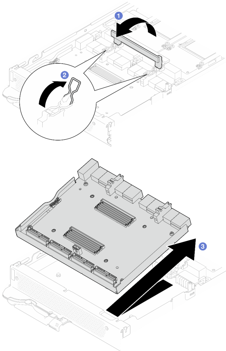
图 327. 卸下载板
