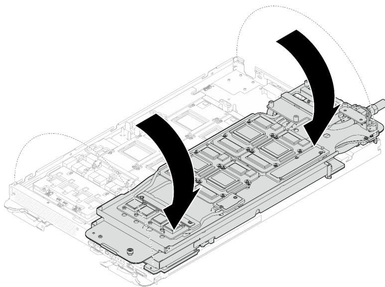
图 346. 将 GPU 节点侧水循环模块折叠到计算节点侧水循环模块上
