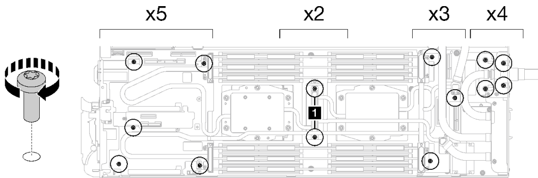
图 218. 安装水循环模块螺钉和快接件螺钉
