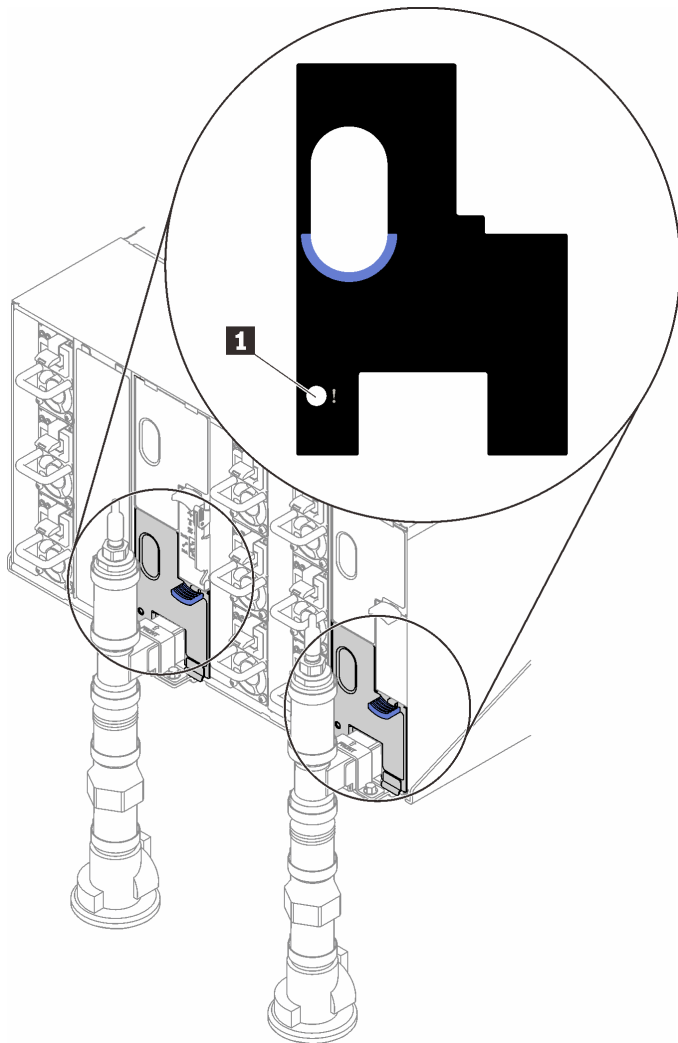
图 477. 液滴传感器 LED
