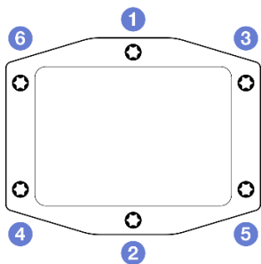
图 259. 处理器冷却板标签
