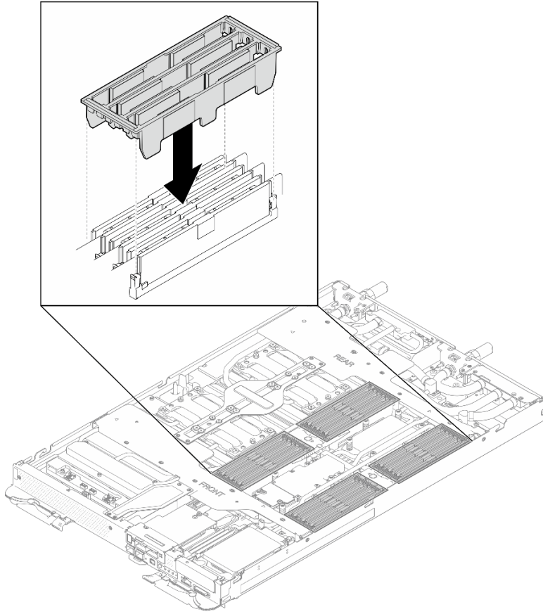
图 170. 安装 DIMM 外盖
