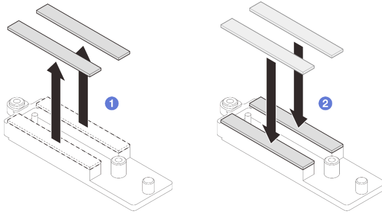
图 308. 更换 VR 导电板油灰垫
