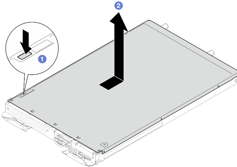
图 18. 卸下托盘外盖
