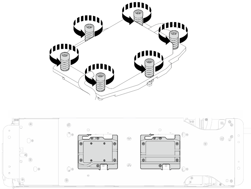
图 260. 卸下处理器冷却板
