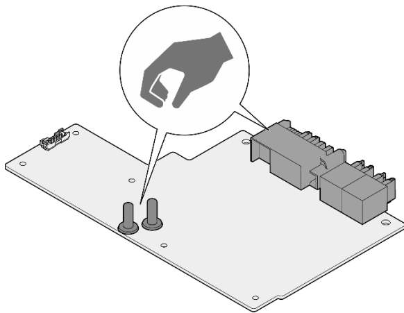
图 393. SD665-N V3 GPU 配电板操作点
