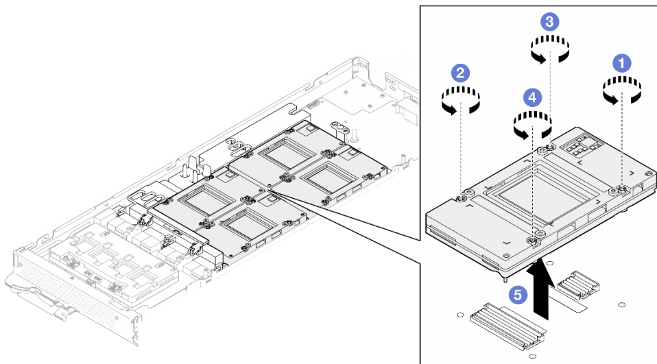
图 349. 卸下 GPU
