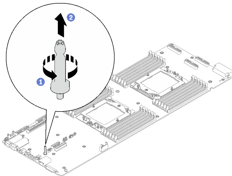
图 287. 卸下导销
