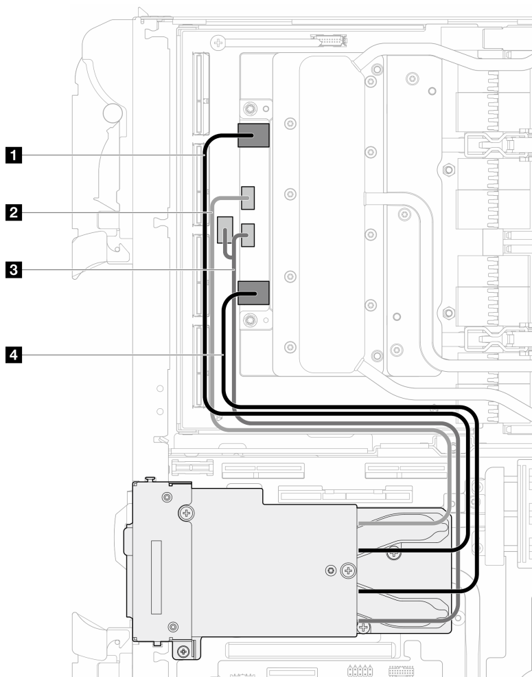
图 183. 从网卡上拔下 OSFP 模块线缆
