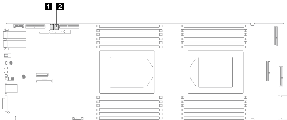
图 9. 计算节点主板上的开关
