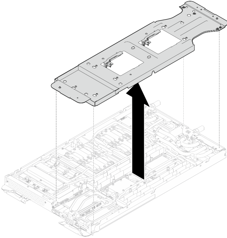
图 65. 卸下水循环模块载板（计算节点）
