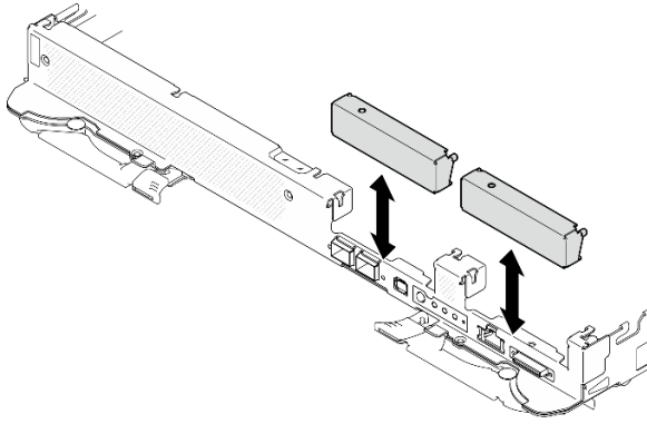
图 151. 安装空挡板填充件
