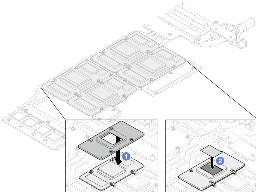
图 447. 更换水循环模块 GPU 冷却板 PCM (GPU 节点)
