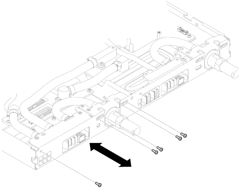
图 279. 安装快接件螺钉 (计算节点)
