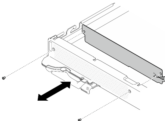
图 462. 安装通风块
