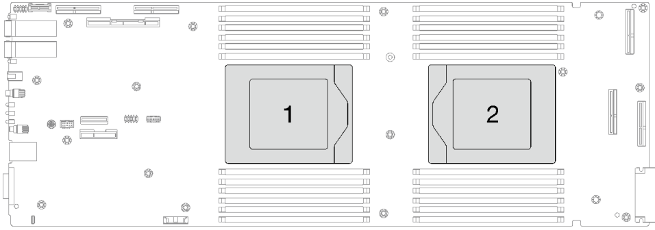
图 236. 处理器位置
