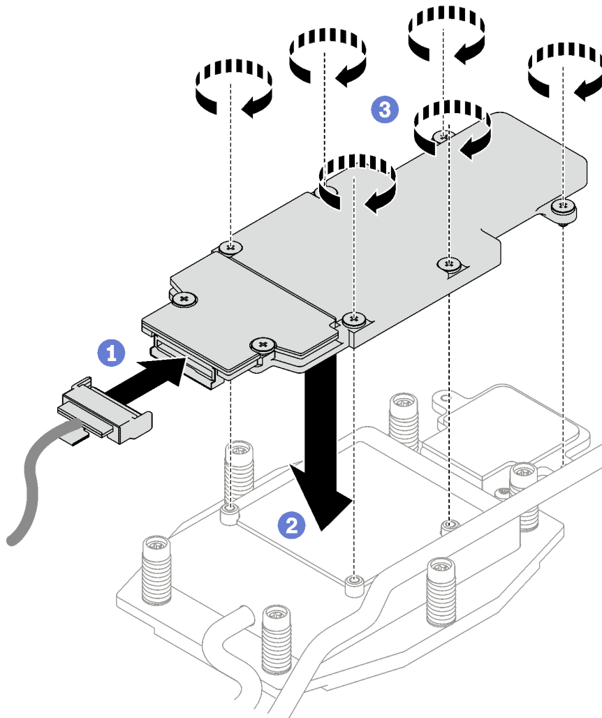
图 163. 安装 M.2 背板组合件
