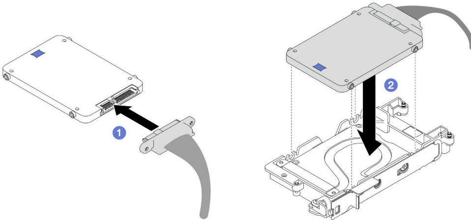
图 127. 安装下方硬盘
