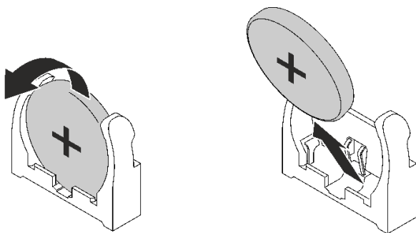
图 93. 卸下 CMOS 电池
