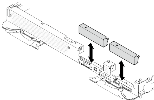
图 136. 卸下空挡板填充件
