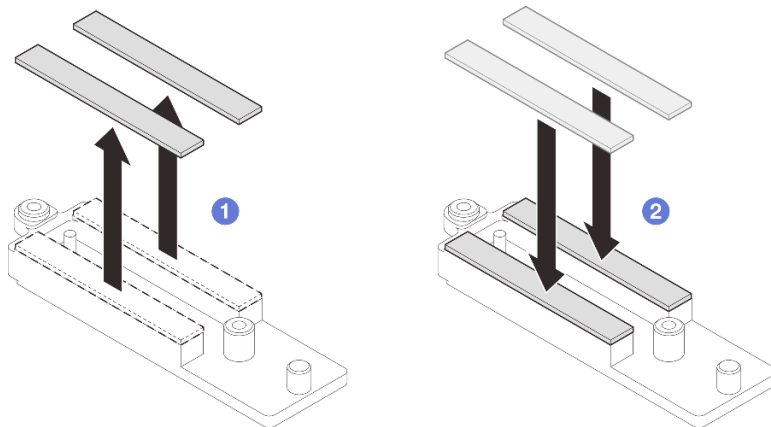
图 318. 更换 VR 导电板油灰垫
