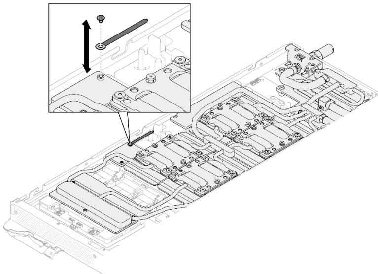
图 25. 取下线缆扎带
