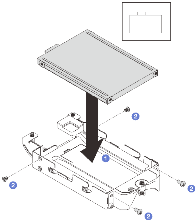
图 147. 安装底部 E3.s 硬盘
