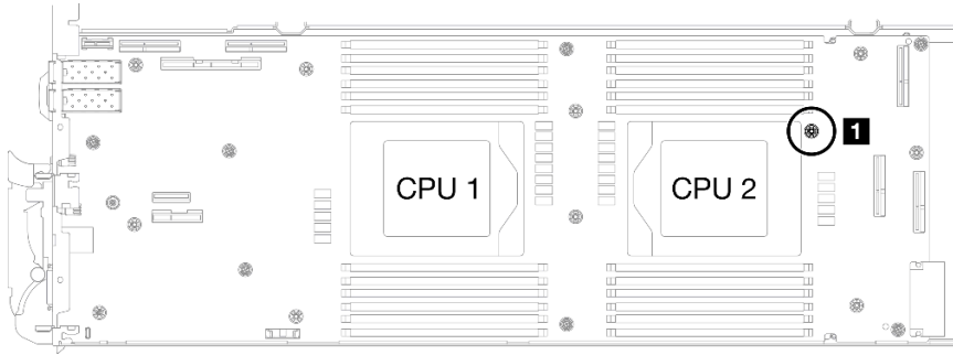
图 296. 屏蔽线缆 4 的螺钉孔的位置
