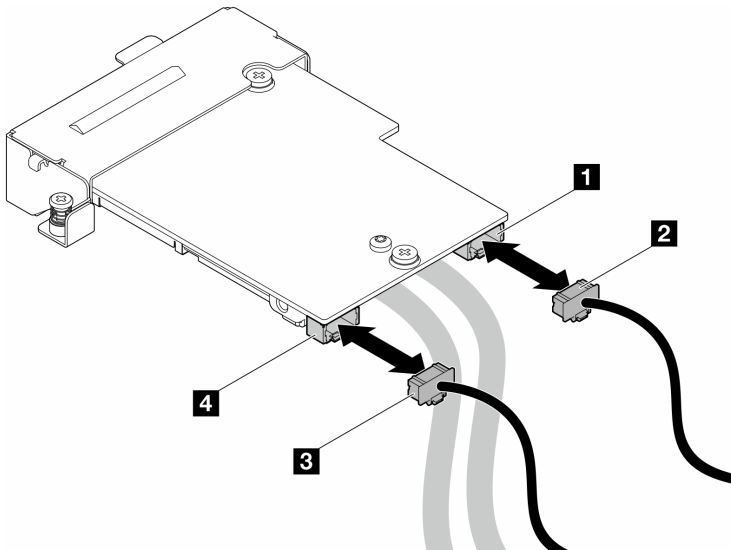
图 188. 安装 OSFP 模块电源线
