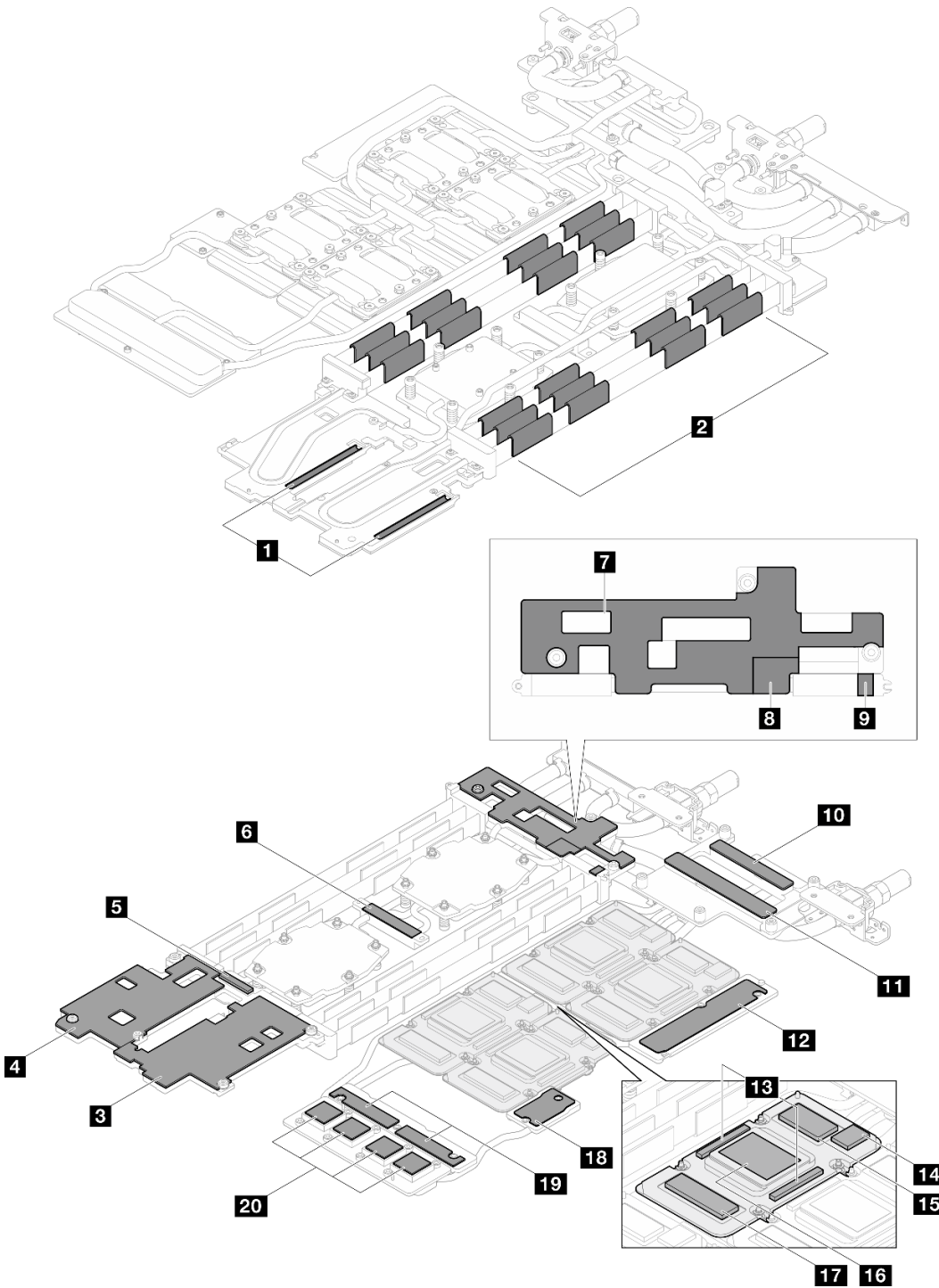
图 15. 水循环模块和 GPU 节点 — 间隙垫/油灰垫的标识和位置
