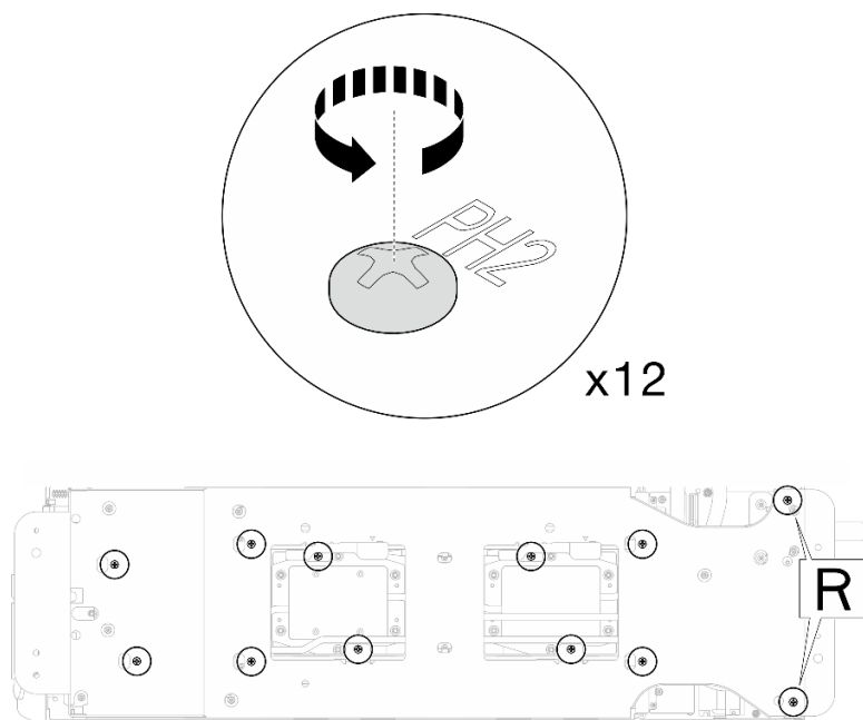
图 262. 安装水循环模块载板螺钉 (计算节点)
