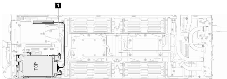
图 179. 拔下硬盘线缆
