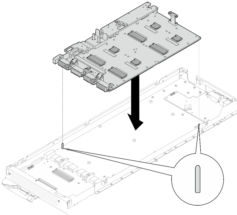
图 374. 安装 GPU 板
