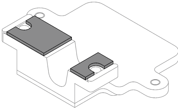
图 160. M.2 背板冷却板（底面）上的油灰垫
