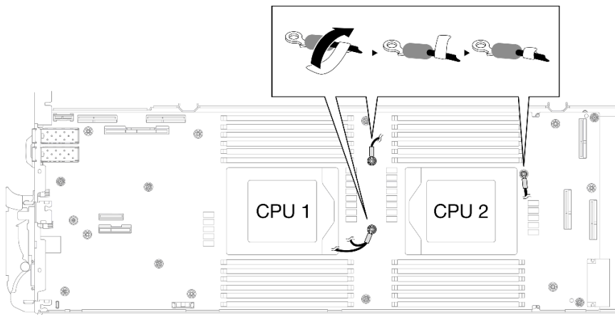
图 298. 将标签缠绕在屏蔽线缆周围
