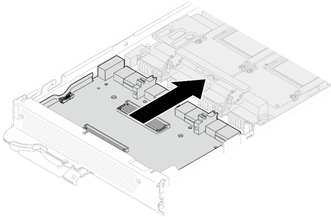
图 390. 将载板连接到 GPU 板
