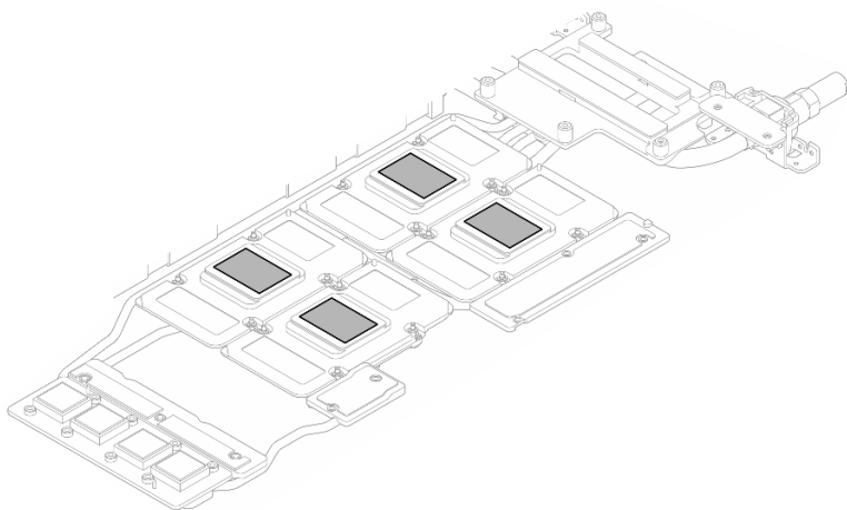
图 441. 清除所有 GPU 上的 PCM
