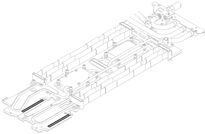
图 210. 水循环模块间隙垫（顶面）
