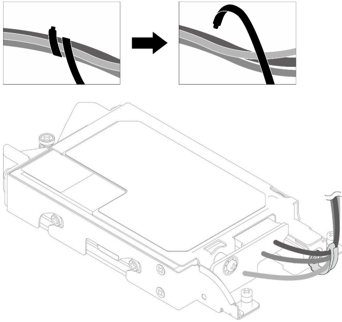
图 137. 从线缆扎带上松开线缆
