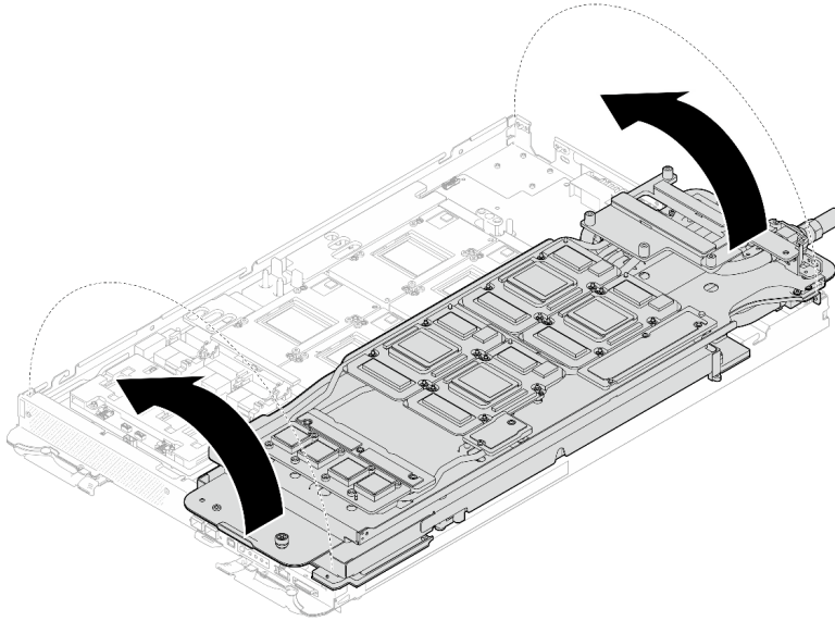
图 356. 将水循环模块展开到 GPU 节点上
