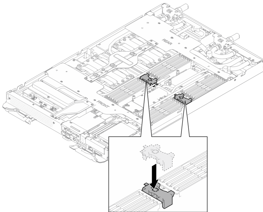
图 98. 安装 DIMM 梳
