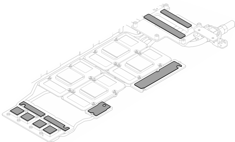
图 442. 清除水循环模块上的油灰垫
