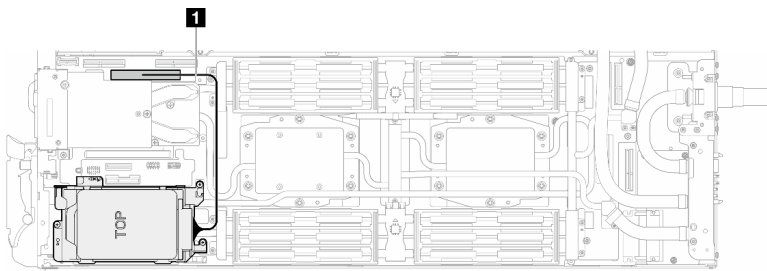
图 119. 连接硬盘仓线缆
