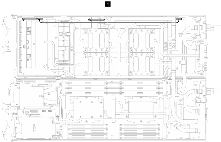
图 24. 拔下载板电源线
