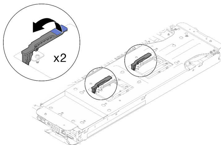
图 263. 将水循环模块与处理器分离
