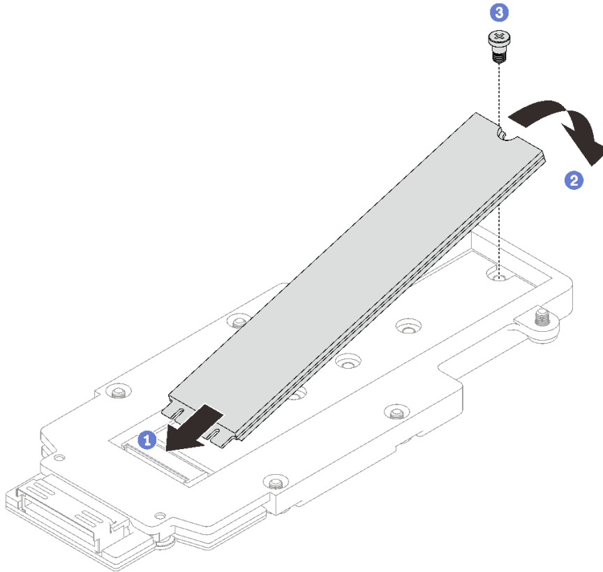
图 159. 安装 M.2 硬盘
