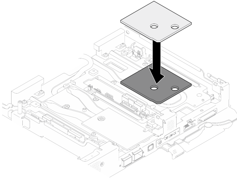
图 131. 更换间隙垫
