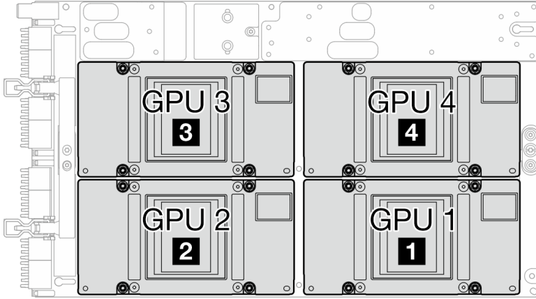
图 5. GPU 编号
