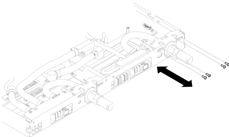
图 422. 安装快接件螺钉（GPU 节点）
