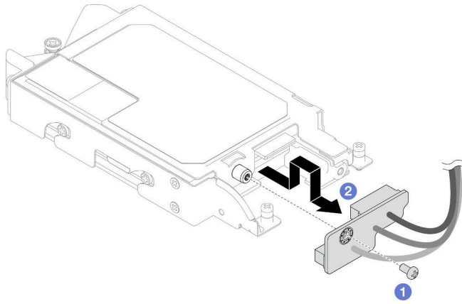
图 139. 卸下 E3.s 硬盘线缆端背板
