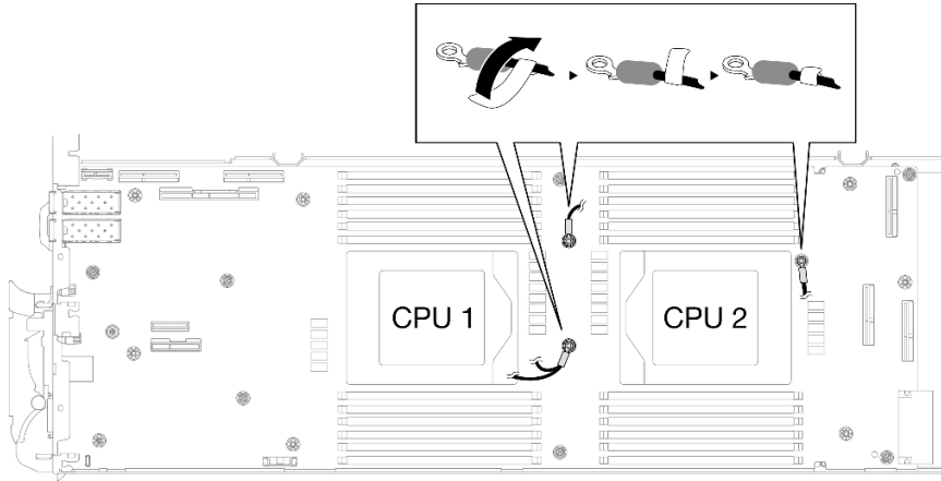
图 315. 将标签缠绕在屏蔽线缆周围
