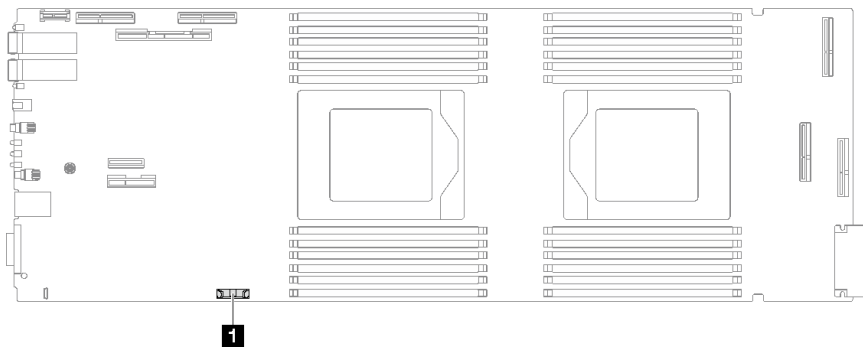
图 92. CMOS 电池位置
