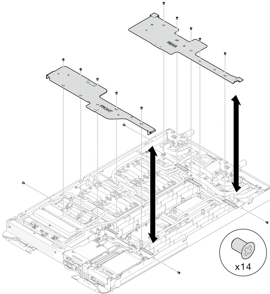
图 21. 卸下正面和背面横梁
