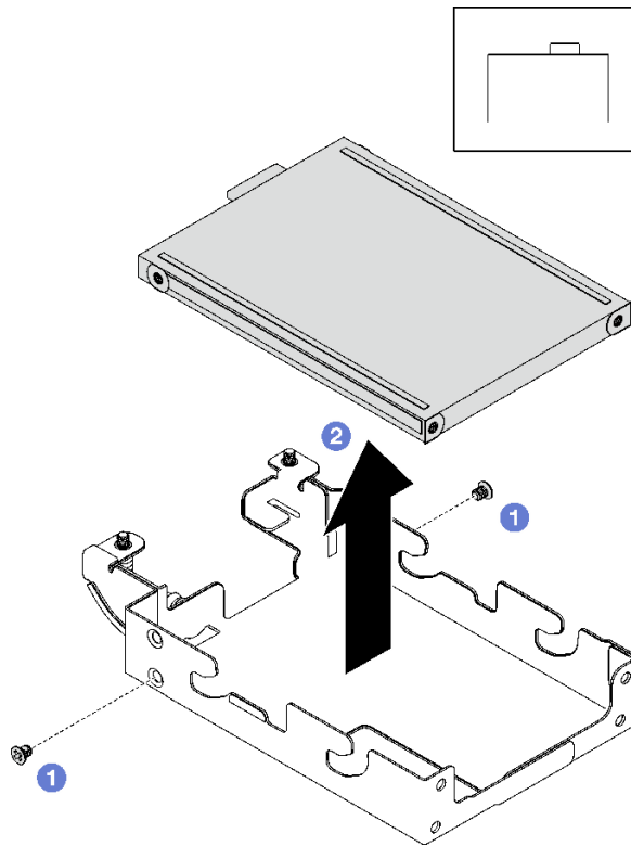
图 142. 卸下顶部 E3.s 硬盘
