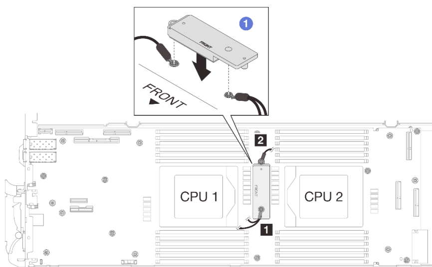
图 293. 将 VR 导电板、屏蔽线缆和主板螺钉孔对齐
