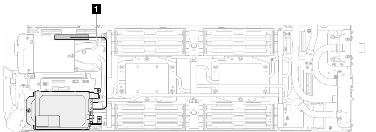
图 180. 拔下 E3.S 硬盘线缆
