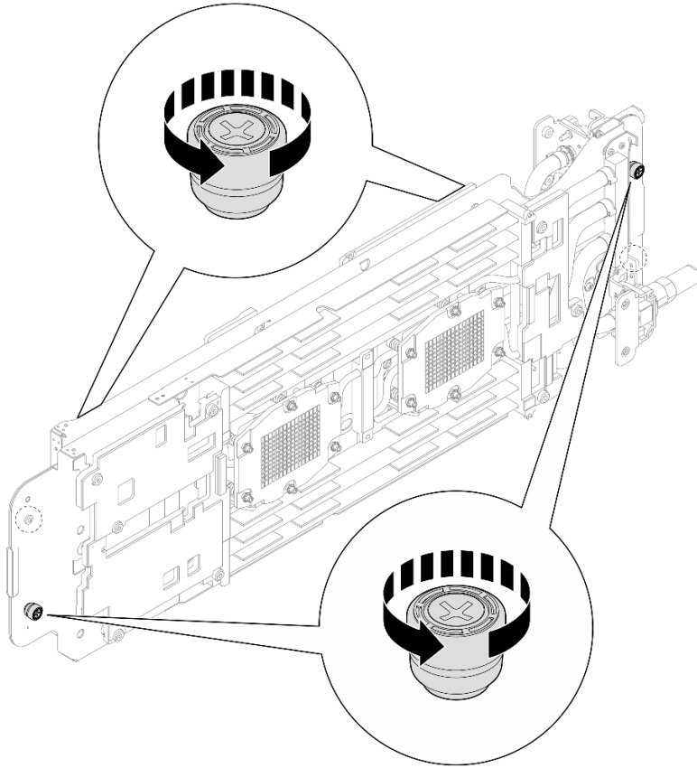
图 55. 拧松水循环模块载板的松不脱指旋螺钉
