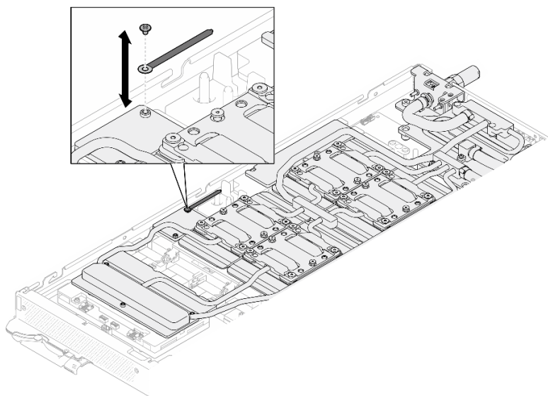
图 458. 安装线缆扎带
