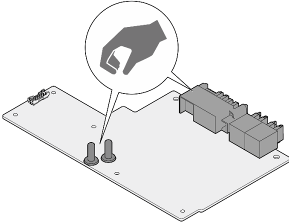
图 411. SD665-N V3 GPU 配电板操作点
