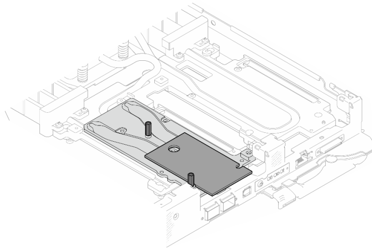
图 187. 更换 OSFP 模块上的油灰垫
