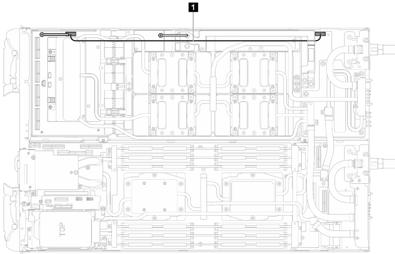
图 394. 拔下载板电源线
