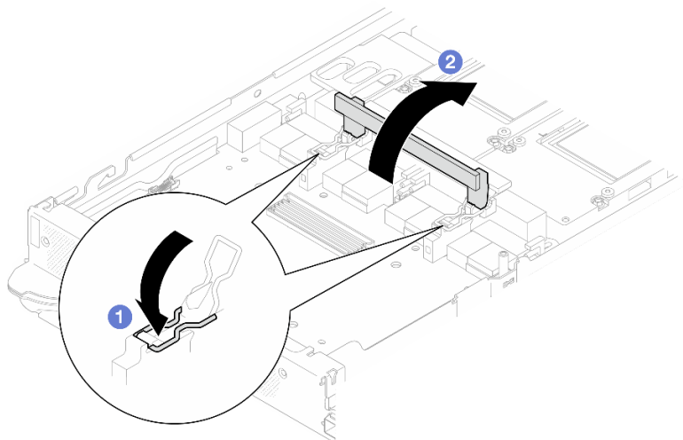
图 330. 将载板固定到 GPU 板上
