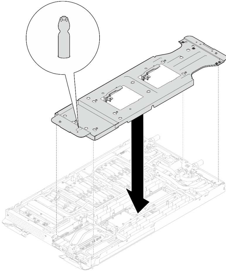
图 231. 安装水循环模块载板（计算节点）
