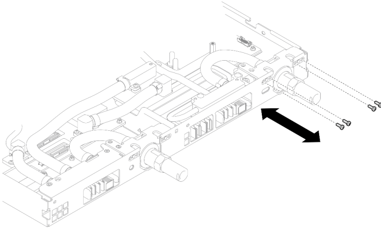
图 455. 安装快接件螺钉 (GPU 节点)
