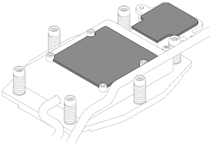
图 162. 处理器冷却板和 M.2 背板冷却板上的油灰垫
