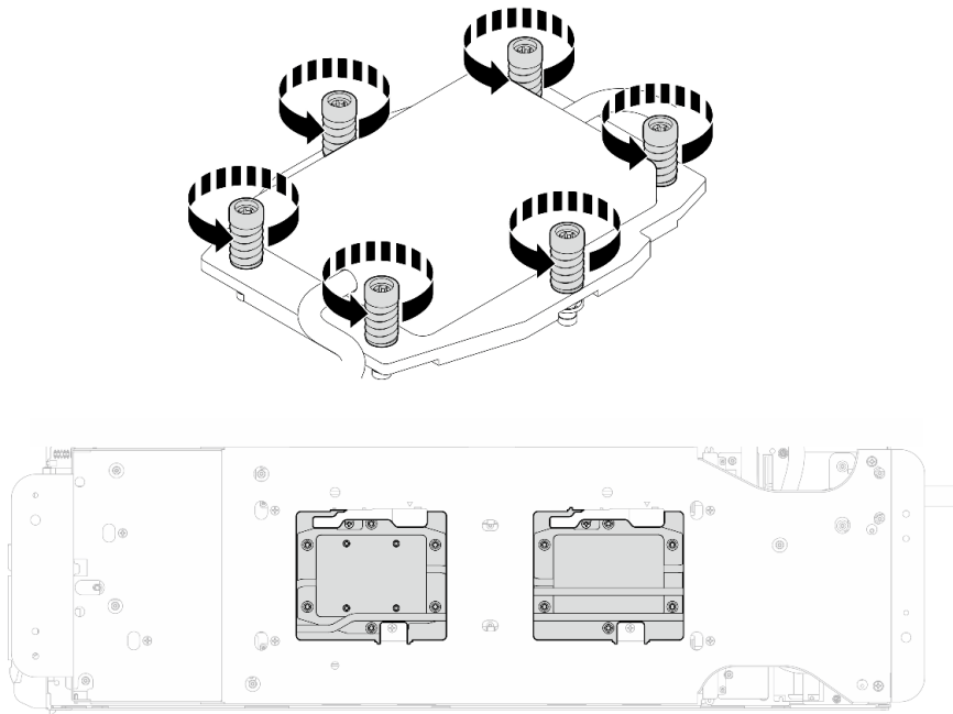
图 46. 卸下处理器冷却板
