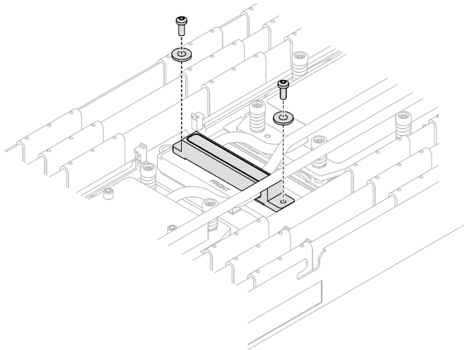
图 43. VR 冷却板螺钉以及垫圈
