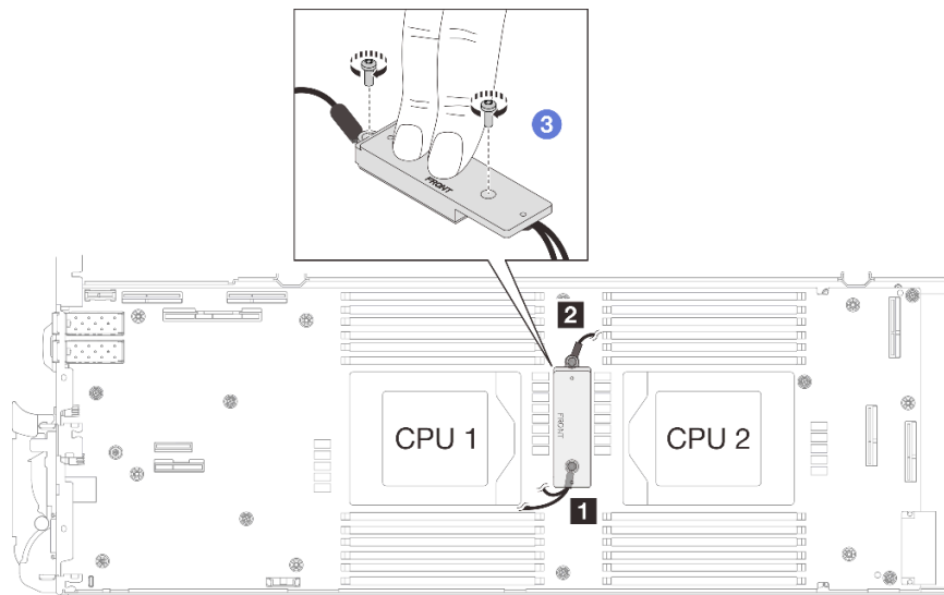
图 295. 连接屏蔽线缆 1/2 和 3
