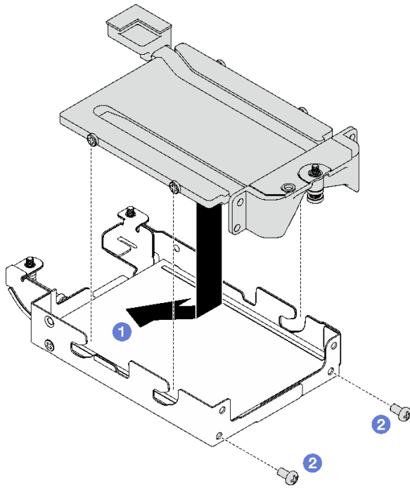
图 146. 安装 E3.s 硬盘导电板
