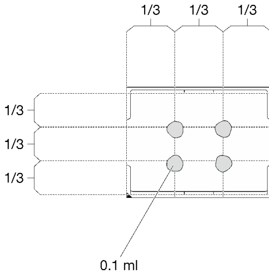
图 267. 涂抹导热油脂
