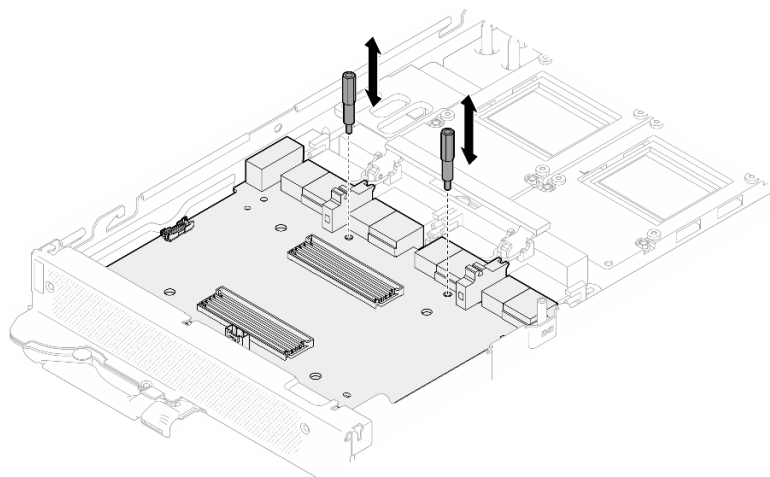
图 331. 安装载板支脚
