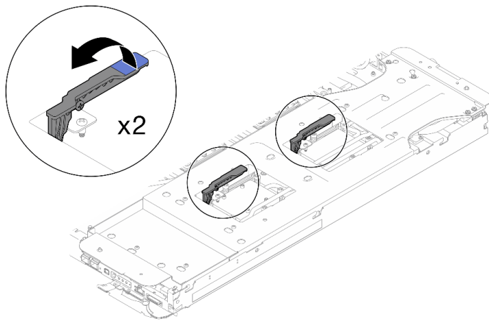
图 233. 将水循环模块与处理器分离
