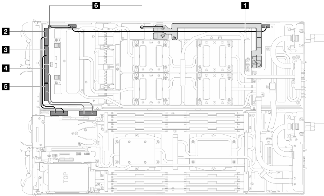
图 465. 单处理器配置线缆布放
