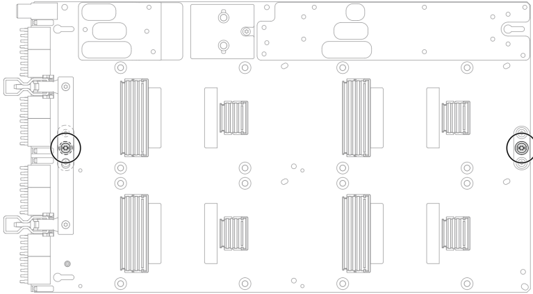
图 370. 卸下 GPU 板 T15 螺钉
