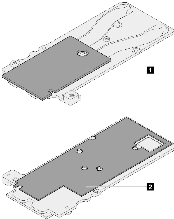
图 70. 更换 OSFP 模块导电板油灰垫
