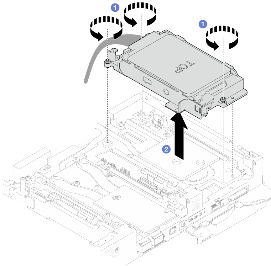
图 102. 卸下双 7 毫米硬盘仓组合件
