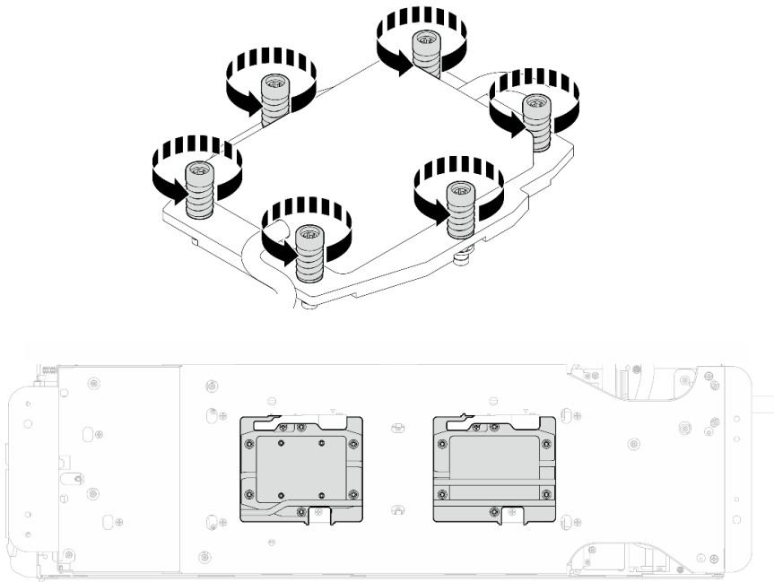
图 230. 卸下处理器冷却板
