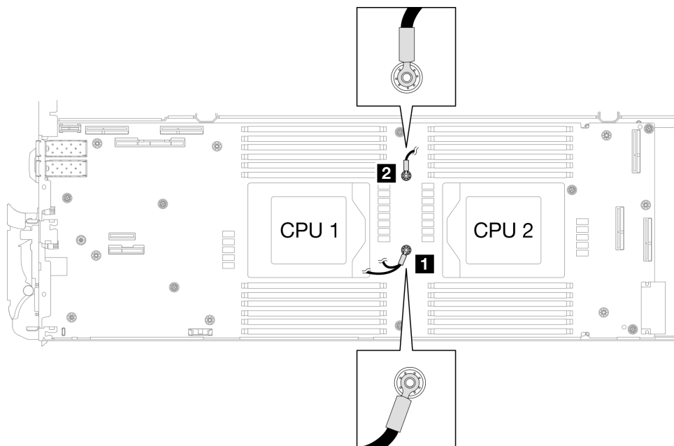
图 292. 将屏蔽线缆 1/2 和屏蔽线缆 3 与螺钉孔对齐
