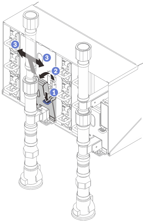
图 478. 卸下下方 EMC 保护罩
