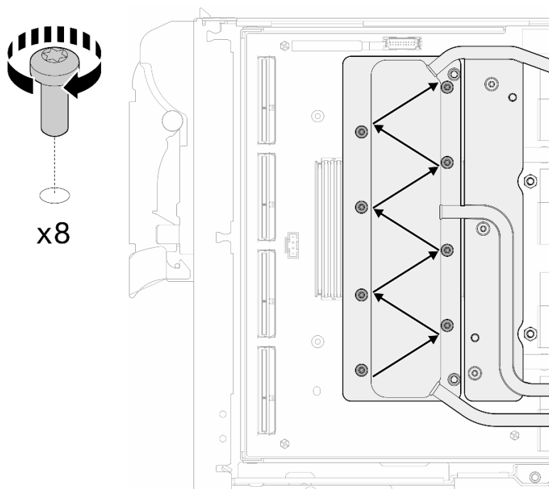
图 76. 安装网卡螺钉
