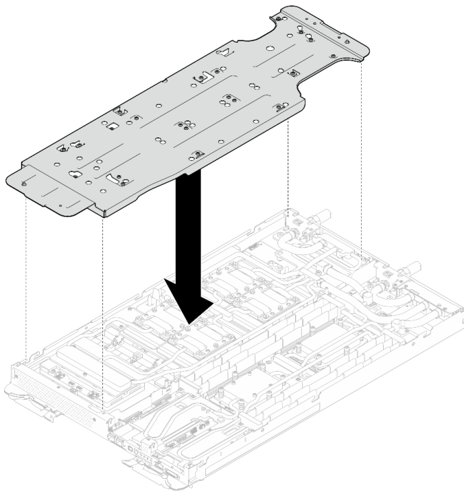
图 34. 安装水循环模块载板 (GPU 节点)
