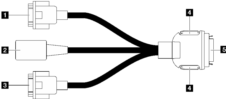
图 6. KVM 分支线缆上的接口和组件
