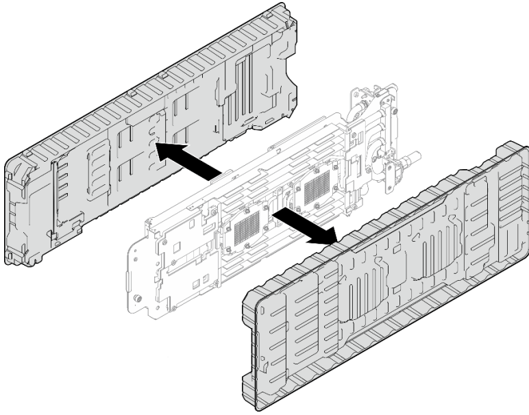
图 239. 卸下塑料油脂外盖
