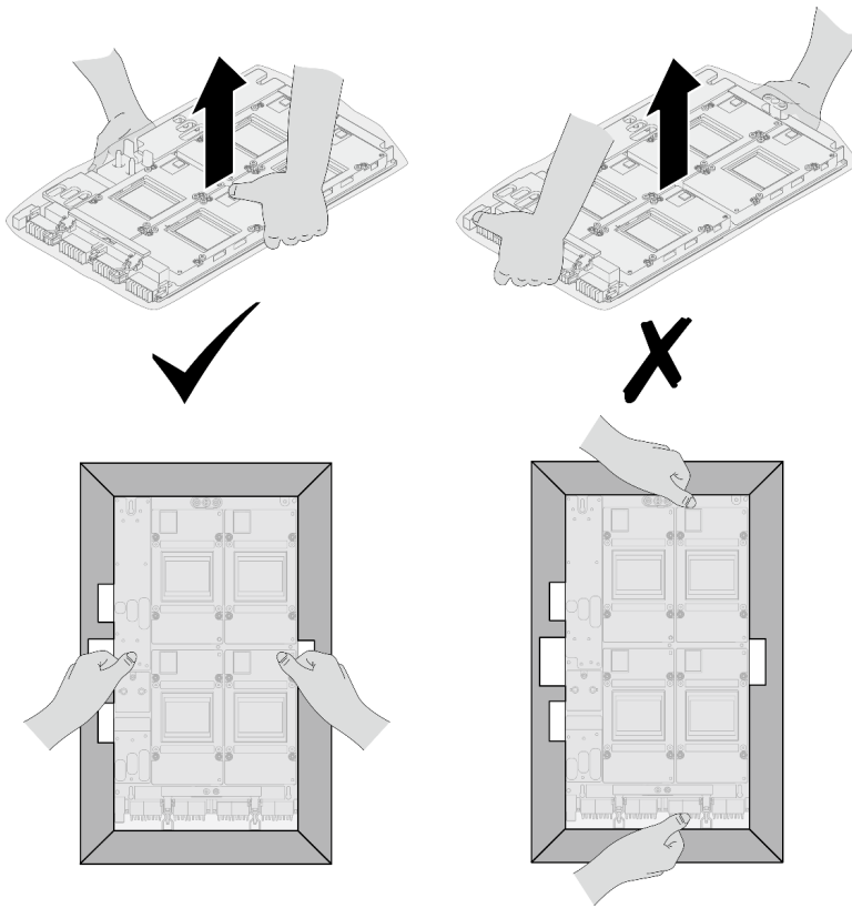
图 385. 从包装盒中取出 GPU 板组合件
