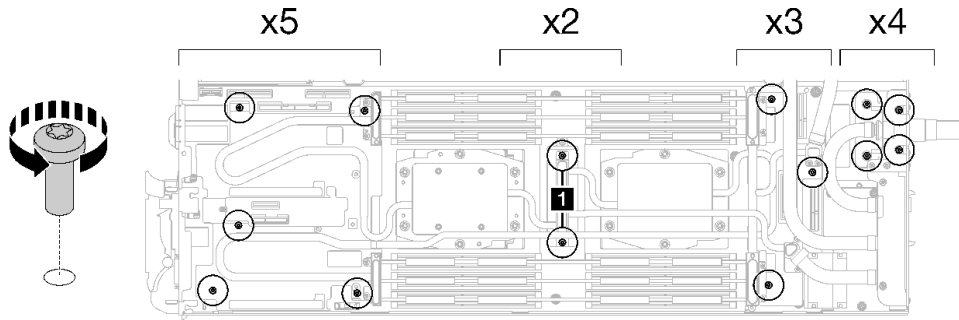
图 228. 卸下水循环模块螺钉
