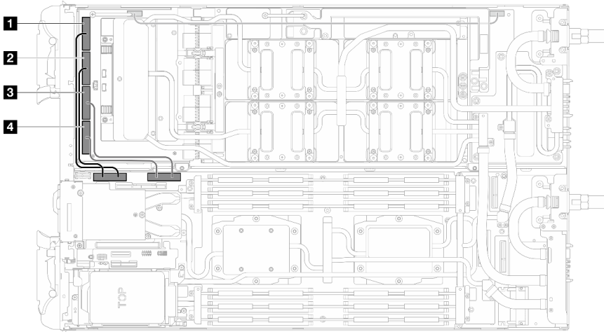
图 181. 单处理器配置 — 拔下所有 MCIO 线缆
