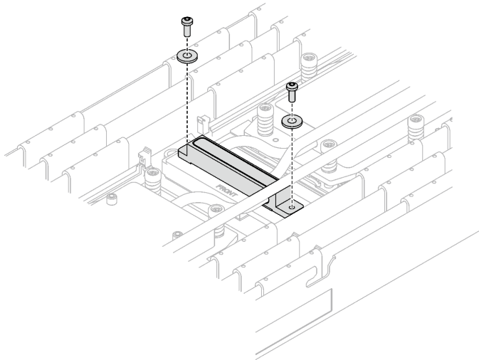
图 198. VR 冷却板螺钉以及垫圈
