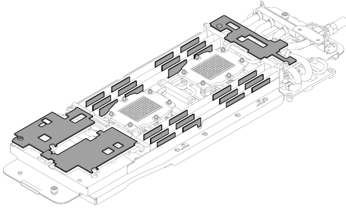
图 57. 水循环模块底面间隙垫（计算节点侧）
