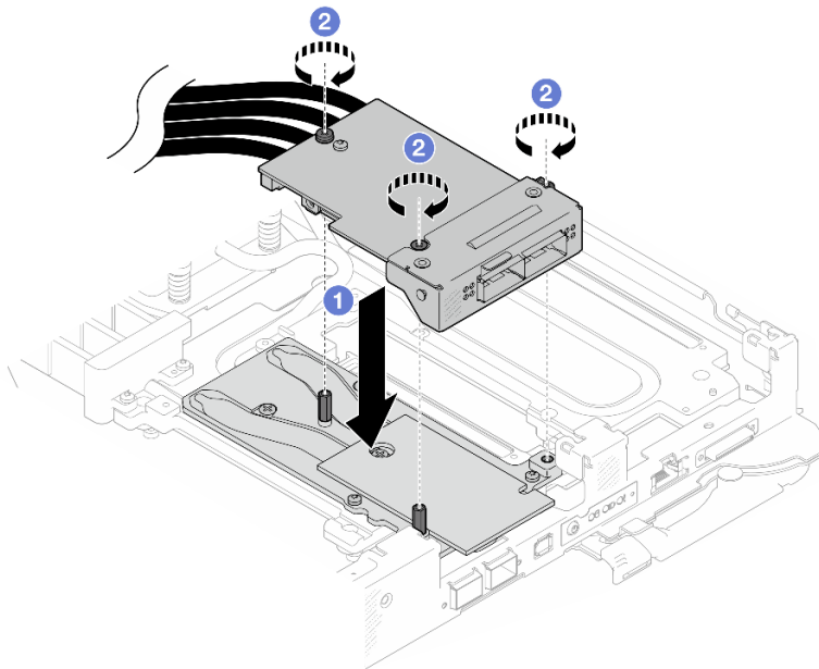
图 189. 安装 OSFP 模块
