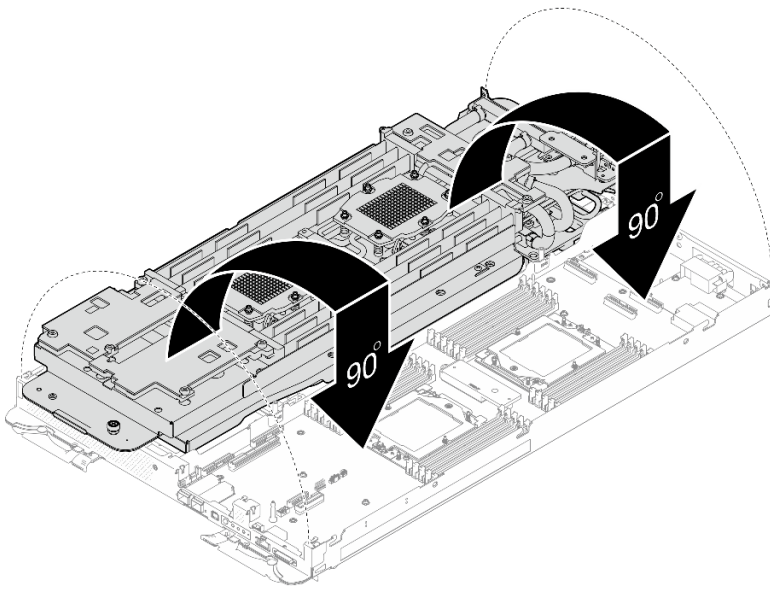
图 273. 安装水循环模块
