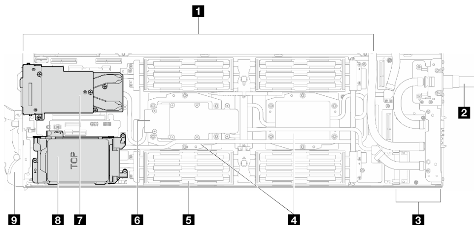
图 3. 计算节点俯视图
