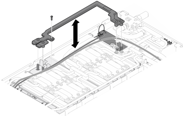
图 322. 卸下汇流条
