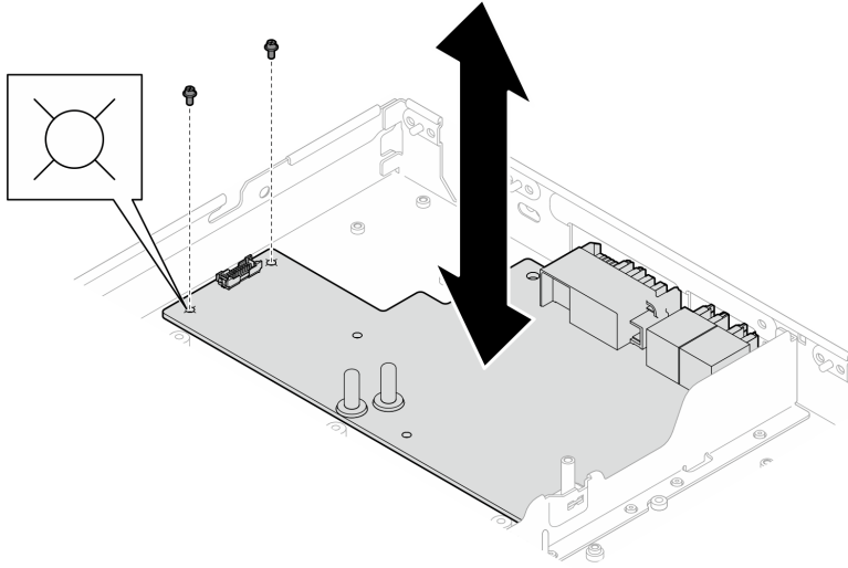
图 409. 卸下 GPU 配电板螺钉
