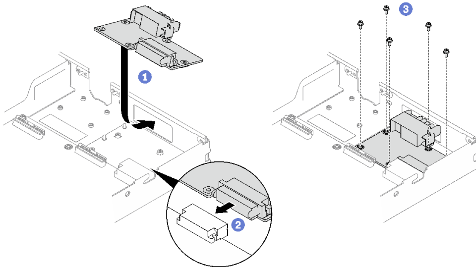
图 207. 安装配电板
