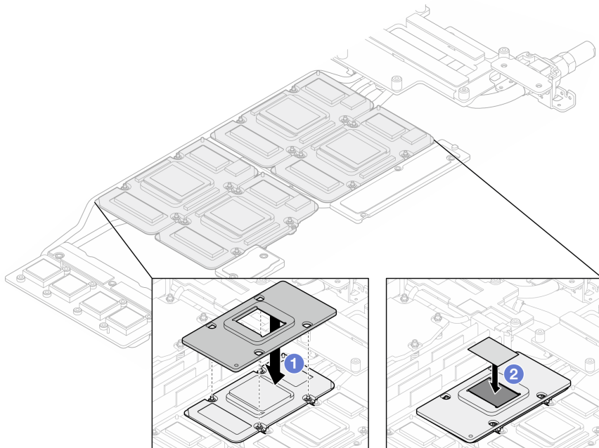
图 59. 更换水循环模块 GPU 冷却板 PCM (GPU 节点)
