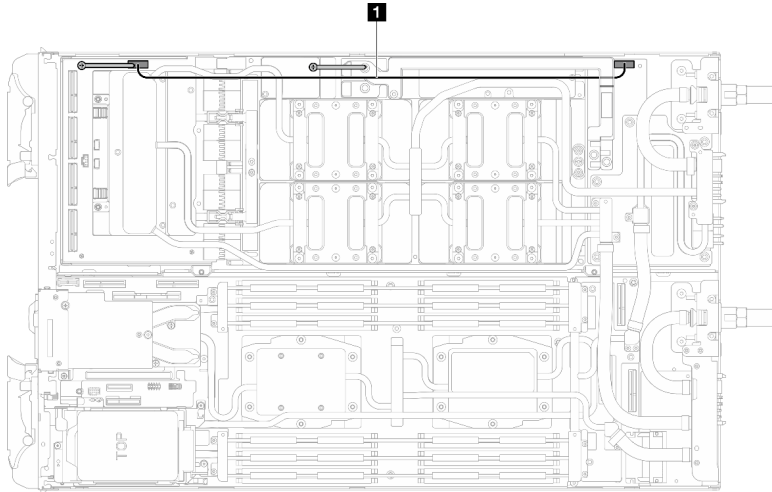
图 81. 连接载板电源线
