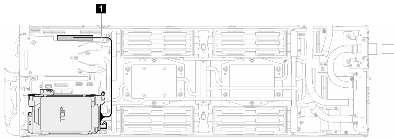
图 100. 拔下硬盘线缆
