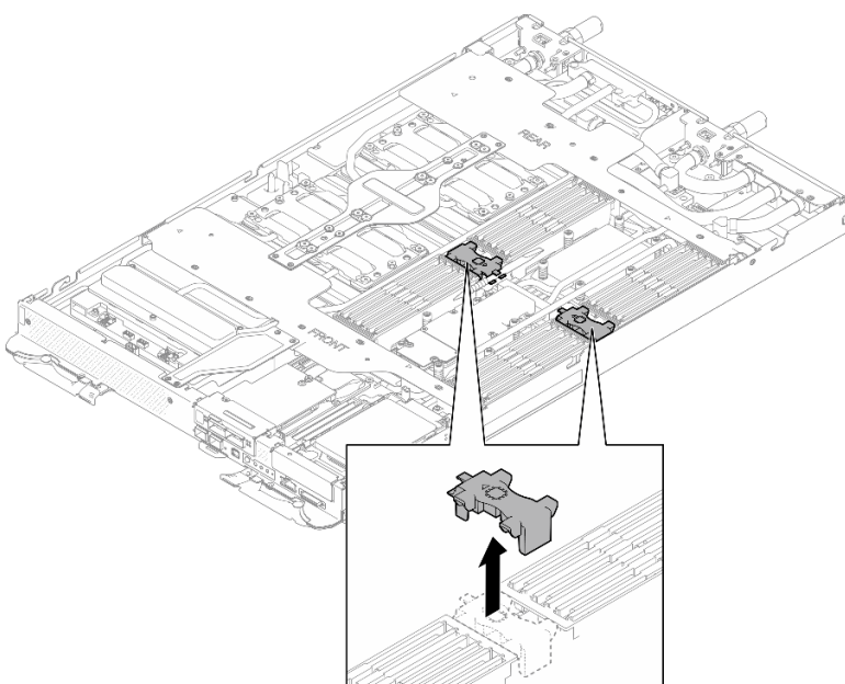
图 97. 卸下 DIMM 梳
