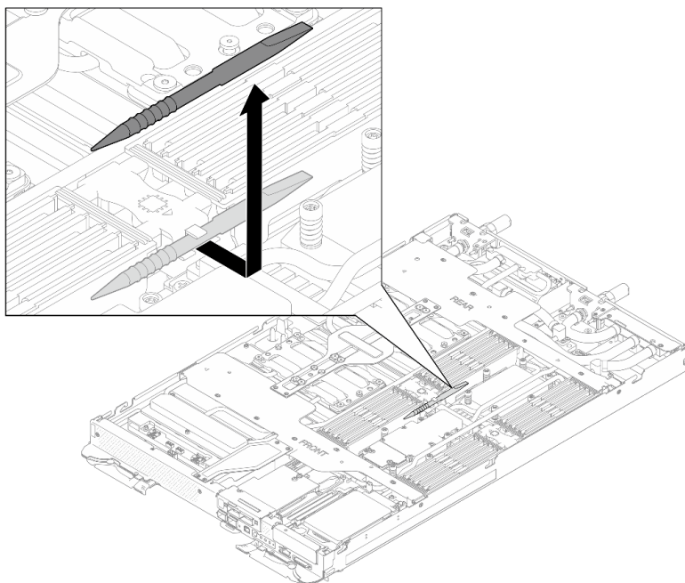
图 96. 卸下内存条工具
