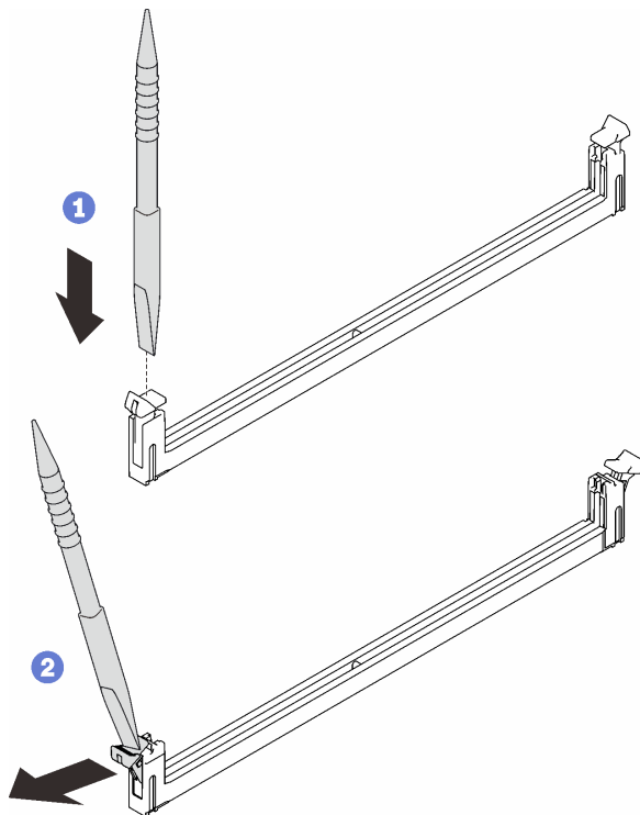
图 175. 按下内存条插槽上的固定夹
