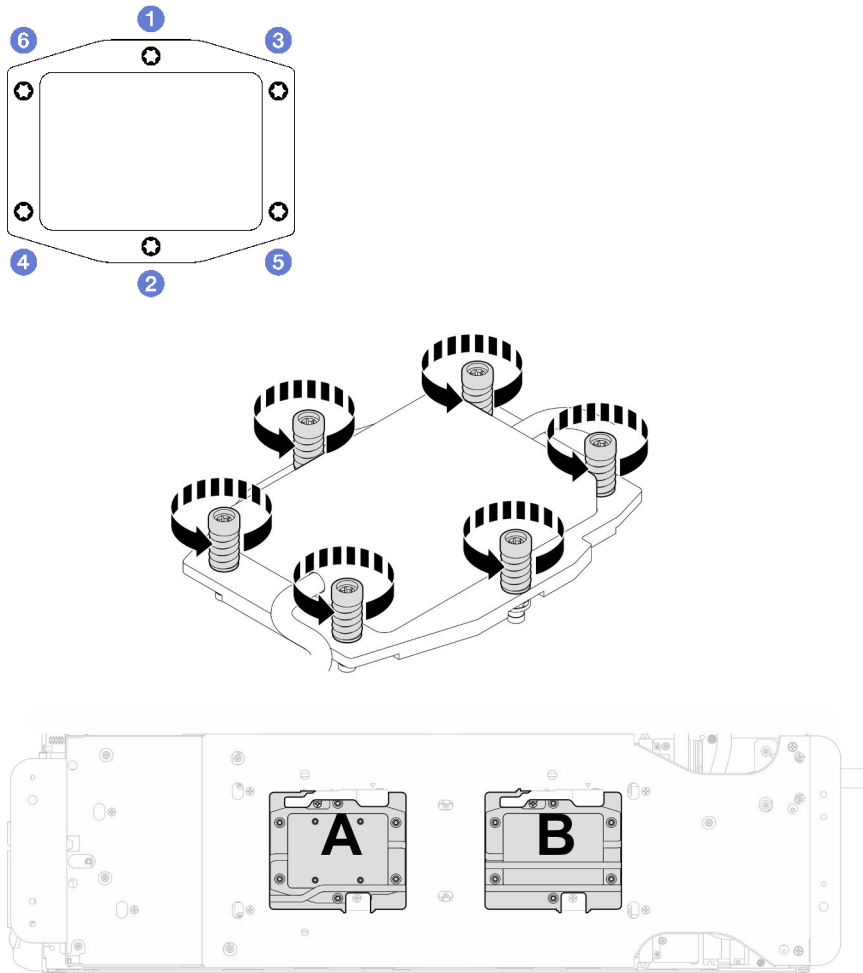
图 216. 安装处理器冷却板
