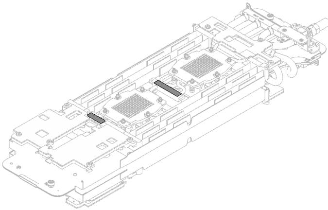
图 211. 水循环模块油灰垫
