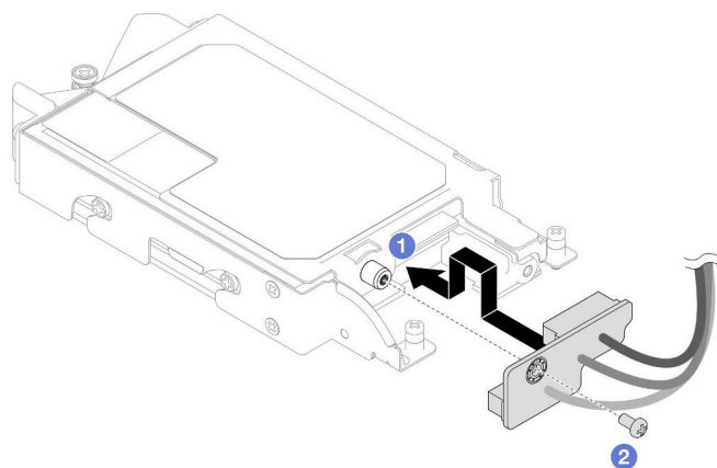
图 148. 安装 E3.s 线缆端背板
