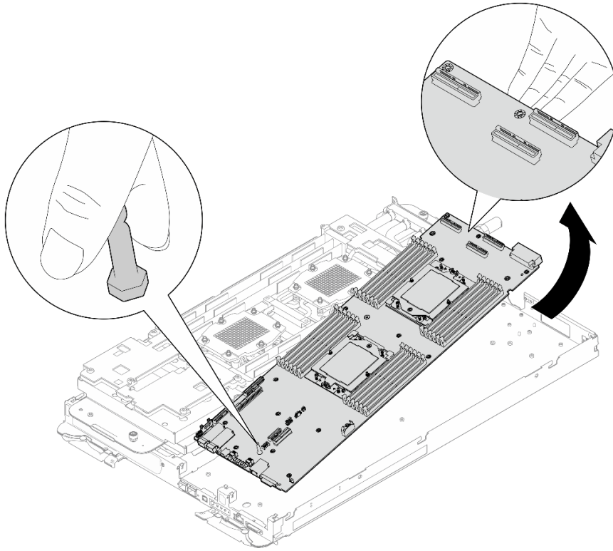
图 286. 卸下主板
