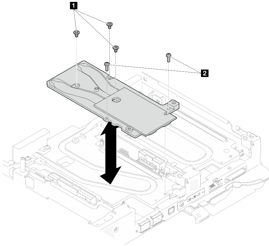
图 255. 卸下 OSFP 模块导电板
