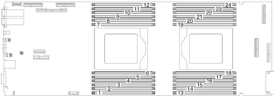
图 165. 内存条插槽位置
