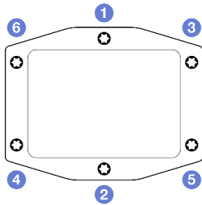
图 229. 处理器冷却板标签
