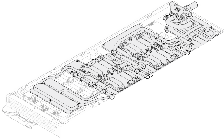
图 32. 用于松开 GPU 冷却板的槽口
