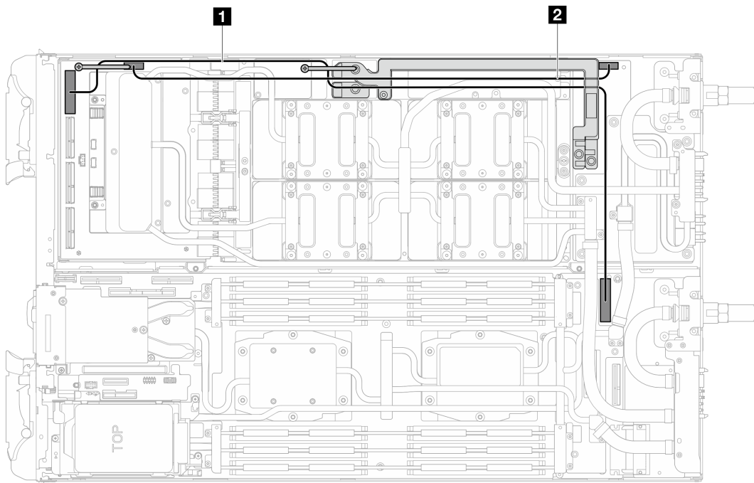
图 323. 布放载板电源线和 MCIO 1 线缆
