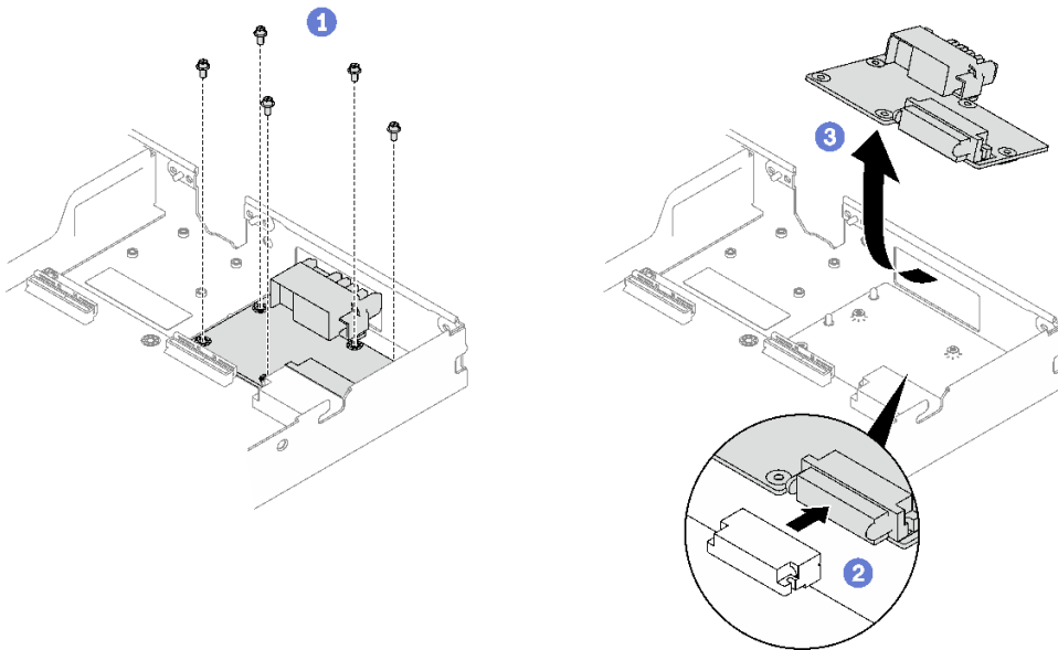
图 206. 卸下配电板
