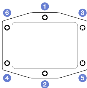
图 200. 处理器冷却板标签
