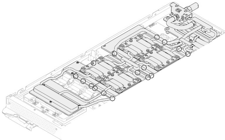
图 342. 用于松开 GPU 冷却板的槽口
