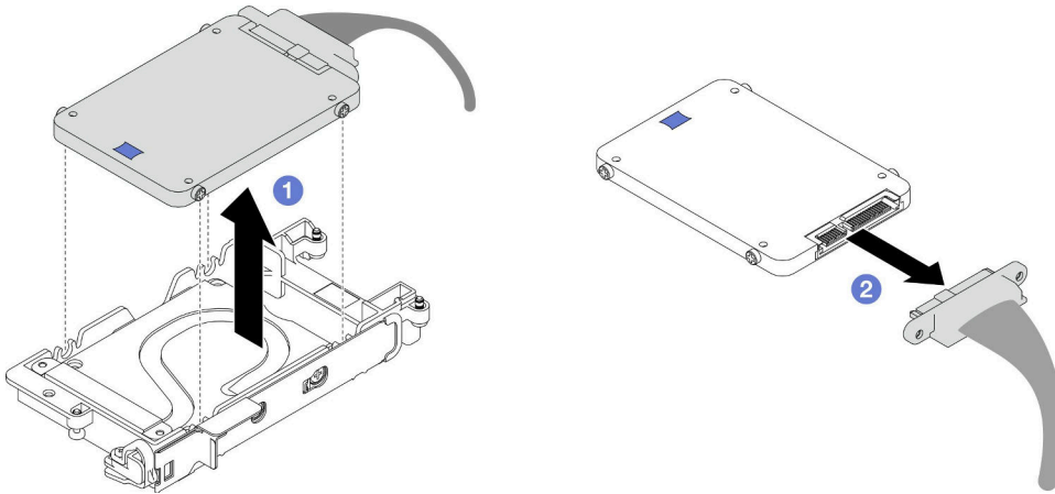
图 124. 卸下方硬盘
