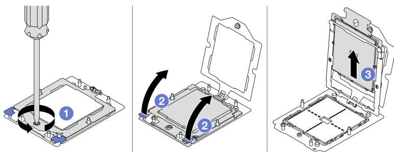
图 235. 卸下处理器
