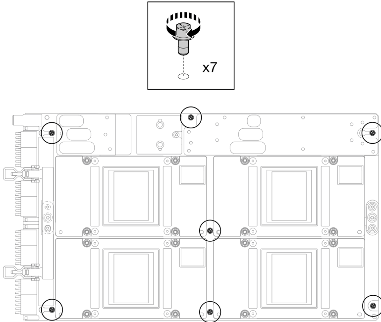
图 388. 将 M3 螺钉安装到 GPU 板组合件上
