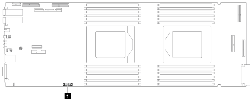
图 94. CMOS 电池位置
