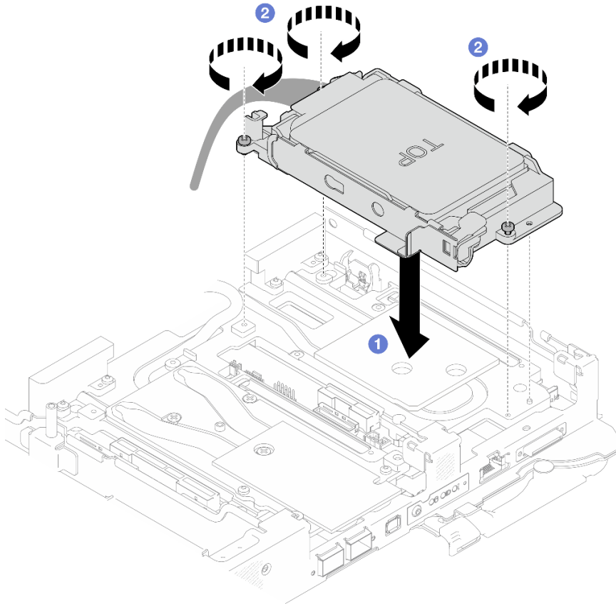
图 118. 安装双 7 毫米硬盘仓组合件
