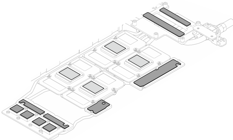
图 60. 更换水循环模块油灰垫 (GPU 节点)
