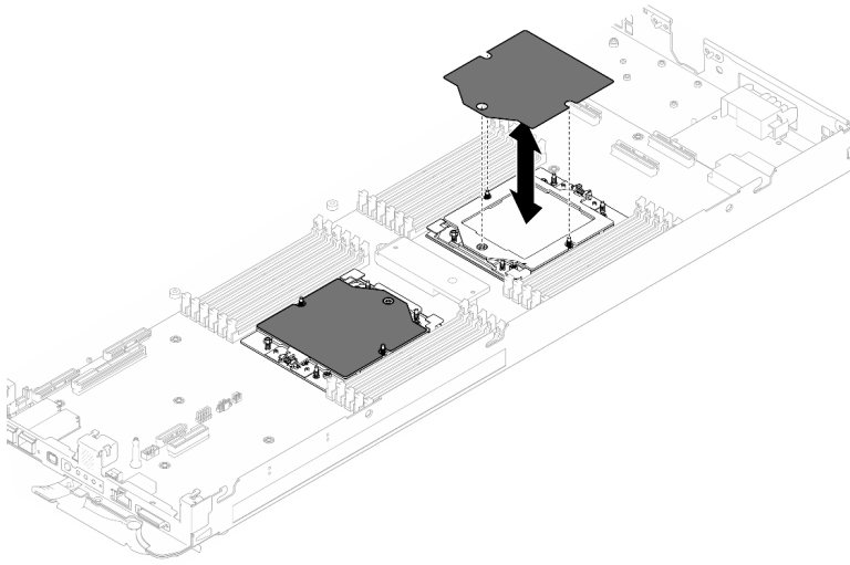
图 266. 贴附处理器插槽保护膜
