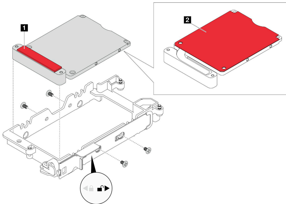
图 110. 安装导电板
