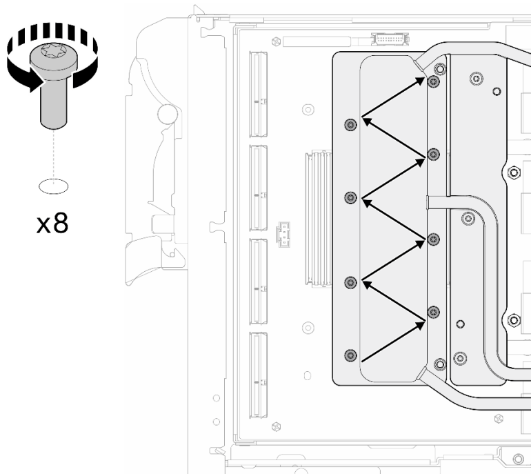
图 29. 卸下网卡螺钉
