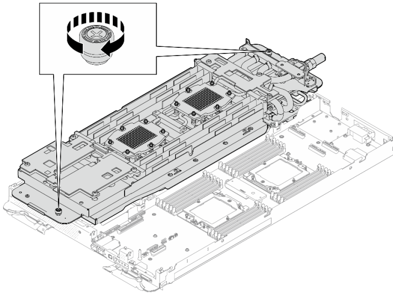
图 51. 拧紧松不脱指旋螺钉
