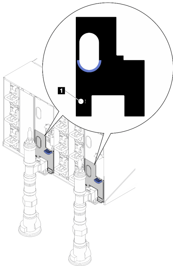
图 474. 液滴传感器 LED
