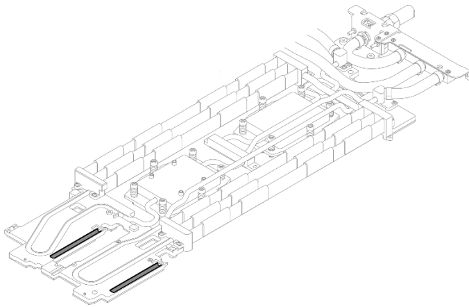
图 58. 水循环模块顶面间隙垫（计算节点侧）
