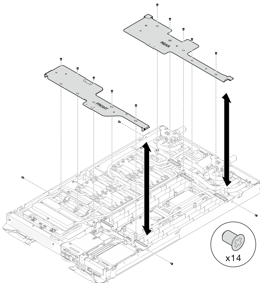
图 22. 安装正面和背面横梁
