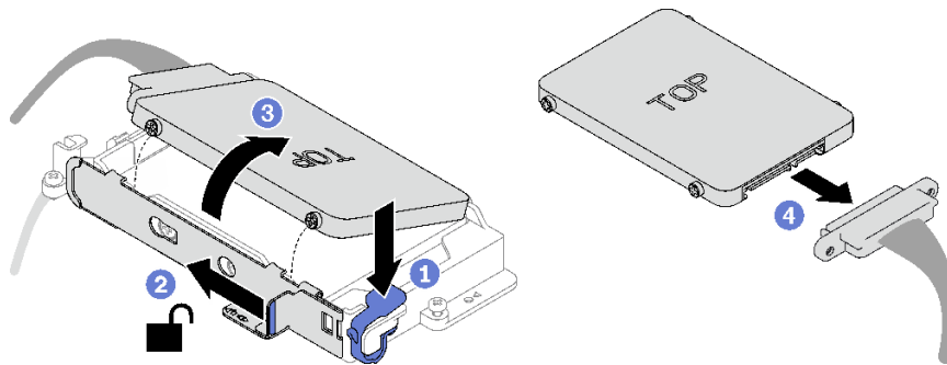
图 105. 卸下上方硬盘
