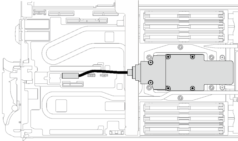
图 164. 安装 M.2 背板组合件线缆
