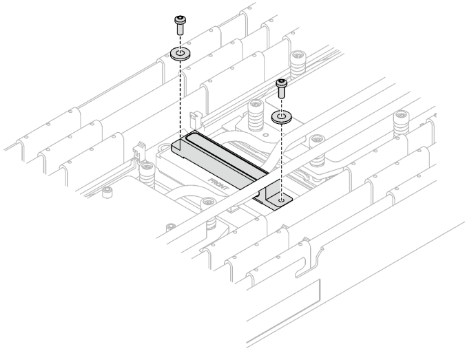
图 277. VR 冷却板螺钉以及垫圈
