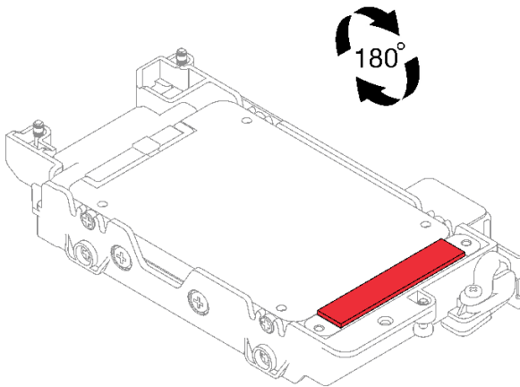
图 114. 间隙垫位置
