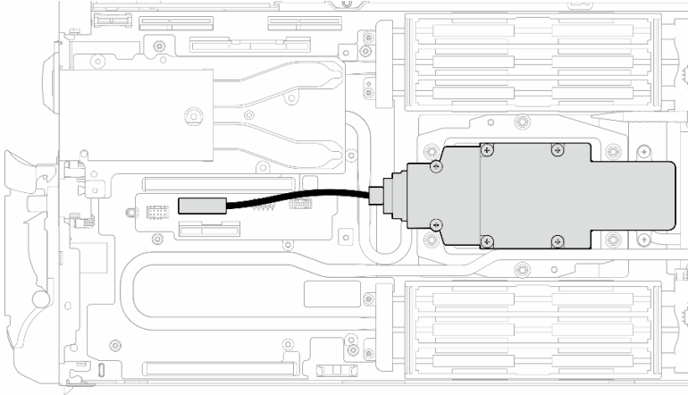
图 155. 拔下 M.2 背板组合件线缆
