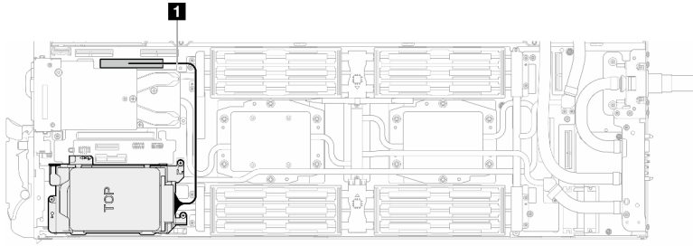
图 120. 拔下硬盘线缆
