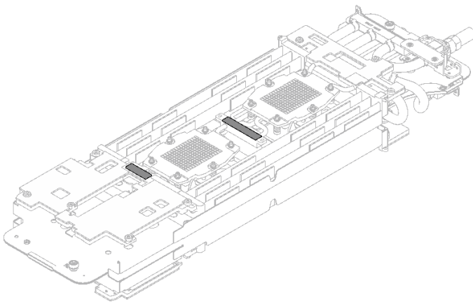
图 242. 水循环模块油灰垫
