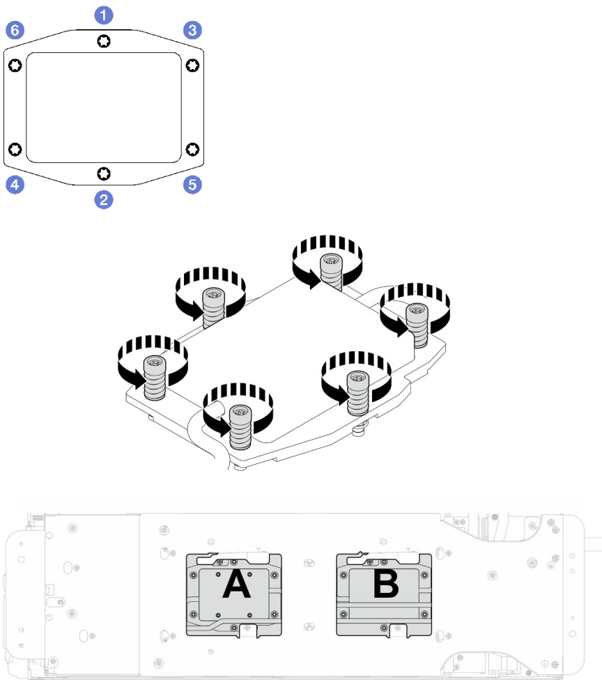
图 247. 安装处理器冷却板
