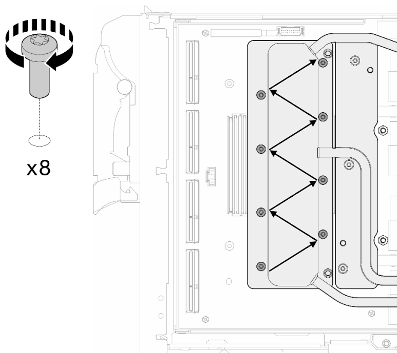
图 421. 安装网卡螺钉
