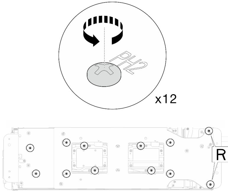
图 203. 安装水循环模块载板螺钉 (计算节点)
