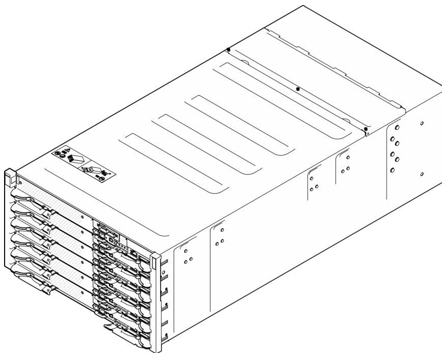
图 1. 装有六个 SD665-N V3 托盘的 DW612S 机柜
