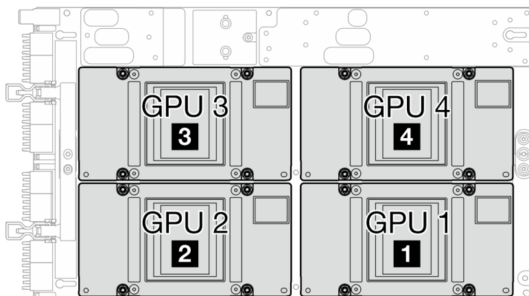
图 10. GPU 编号
