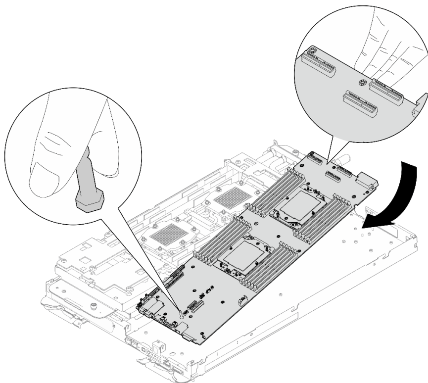
图 289. 安装主板
