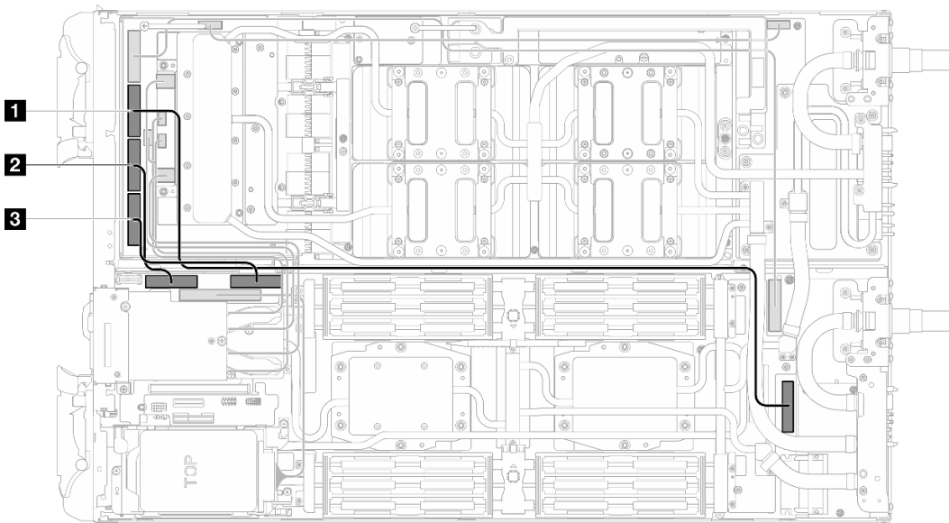
图 182. 双处理器配置 — 拔下 MCIO 2、MCIO 3 和 MCIO 4 线缆
