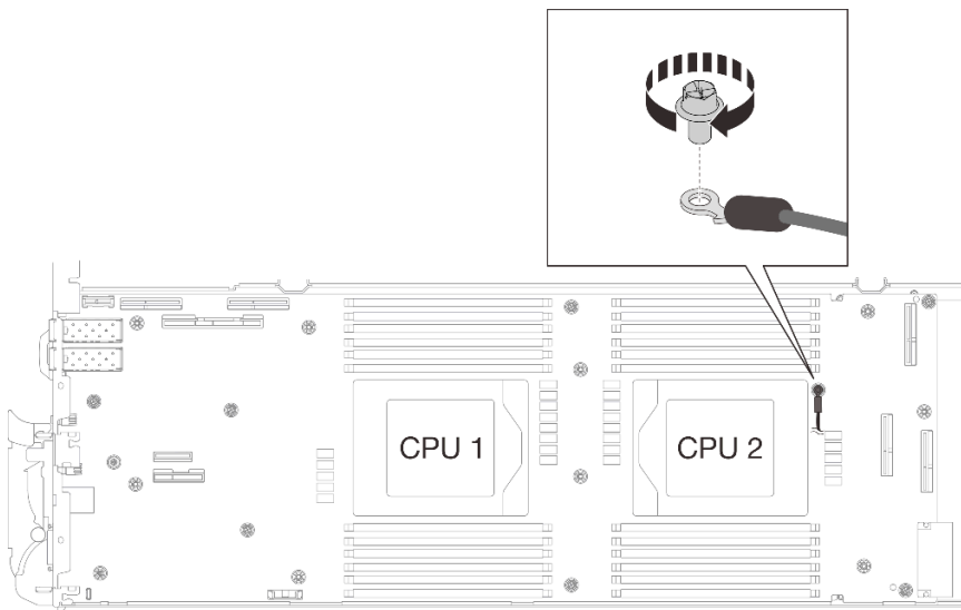
图 297. 连接屏蔽罩线缆 4
