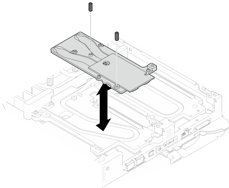
图 224. 卸下 OSFP 模块导电板六角螺钉
