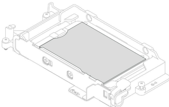
图 125. 安装导电板间隙垫
