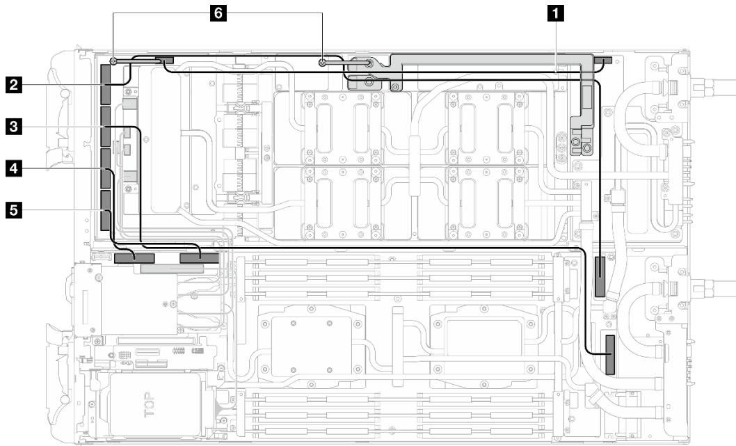
图 466. 双处理器配置线缆布放
