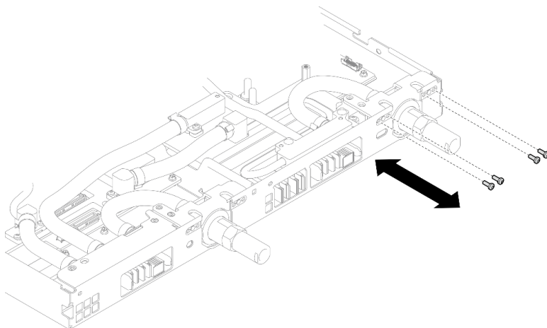
图 361. 安装快接件螺钉 (GPU 节点)
