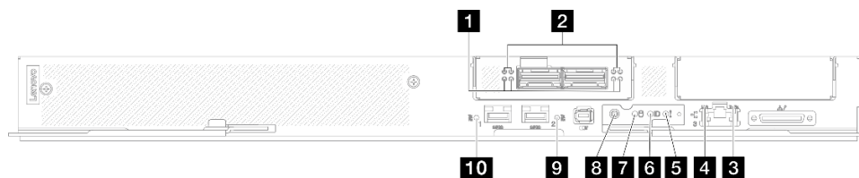
图 470. SD665-N V3 托盘正面 LED
