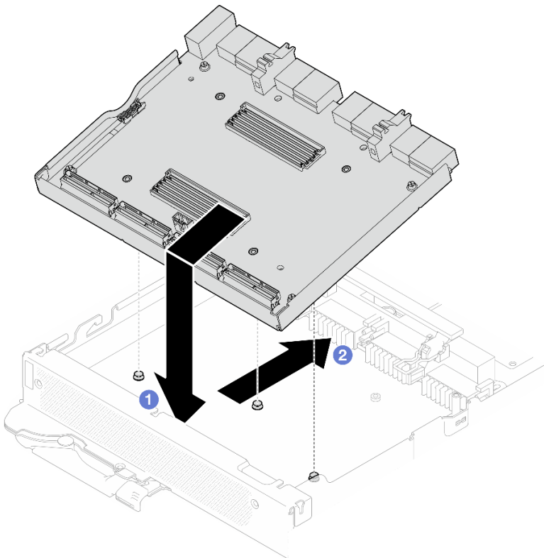
图 329. 安装载板
