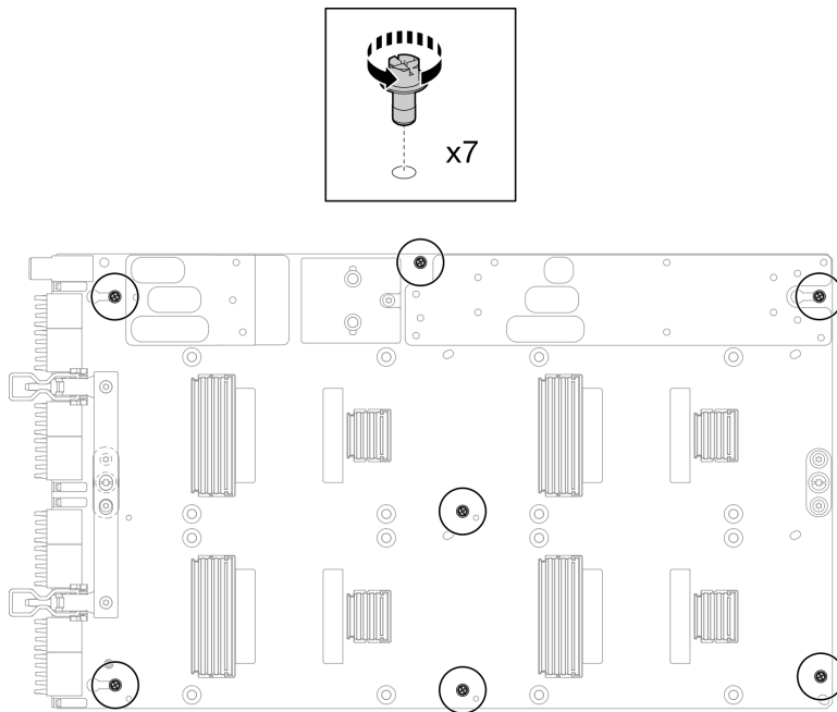
图 369. 卸下 GPU 板 M3 螺钉
