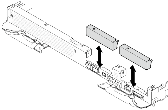
图 122. 卸下空挡板填充件
