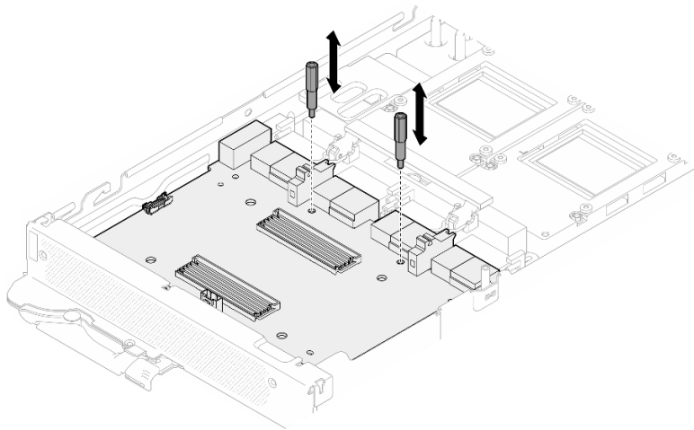
图 326. 卸下载板支脚
