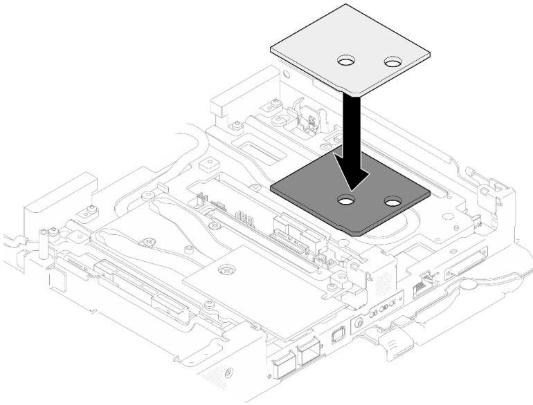
图 116. 更换间隙垫
