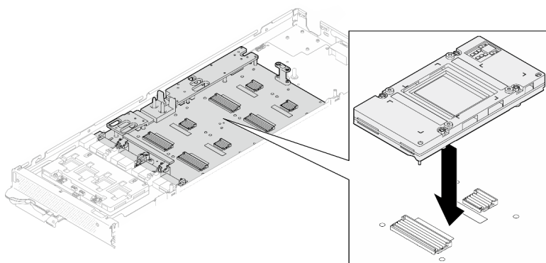
图 351. 安装 GPU
