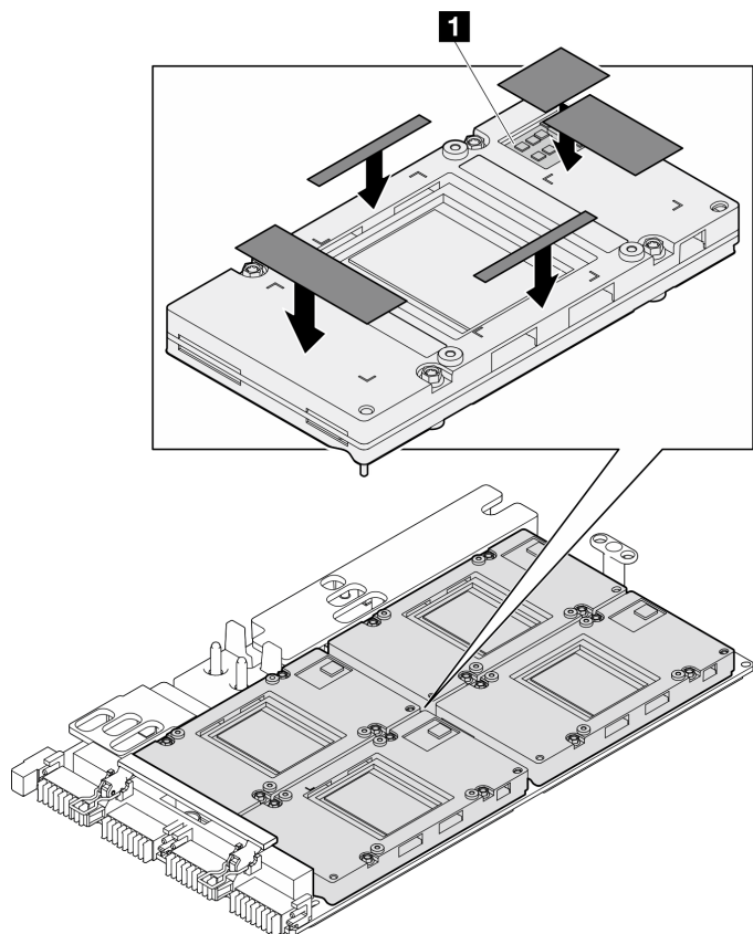
图 449. 更换 GPU 油灰垫
