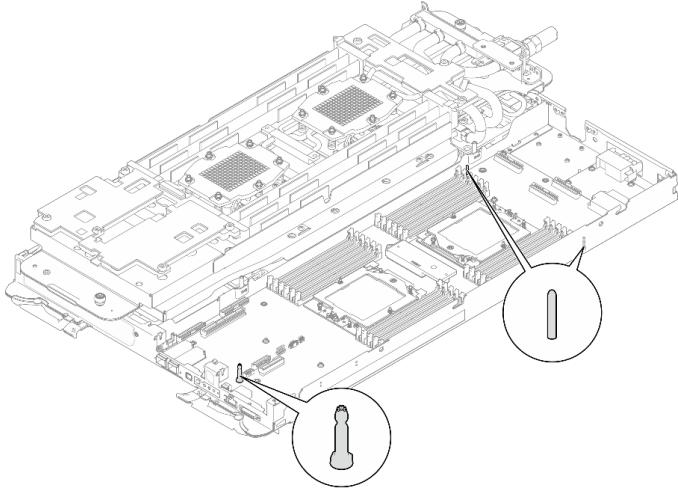
图 272. 计算节点上的导销
