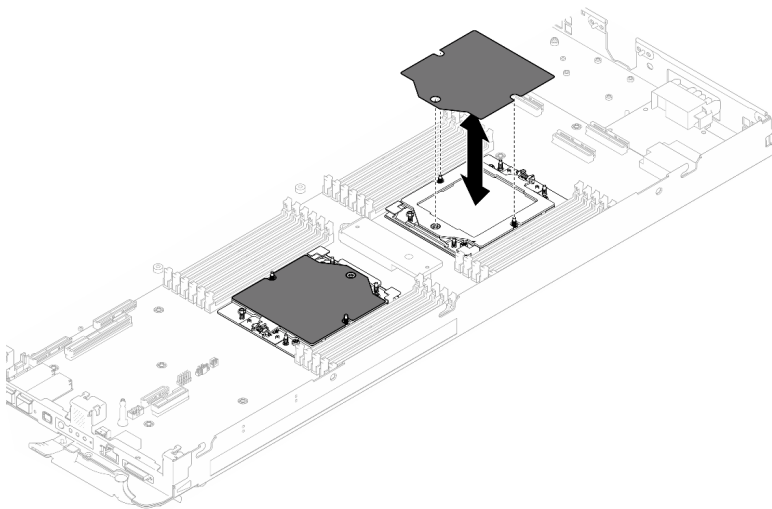
图 265. 撕下处理器插槽保护膜
