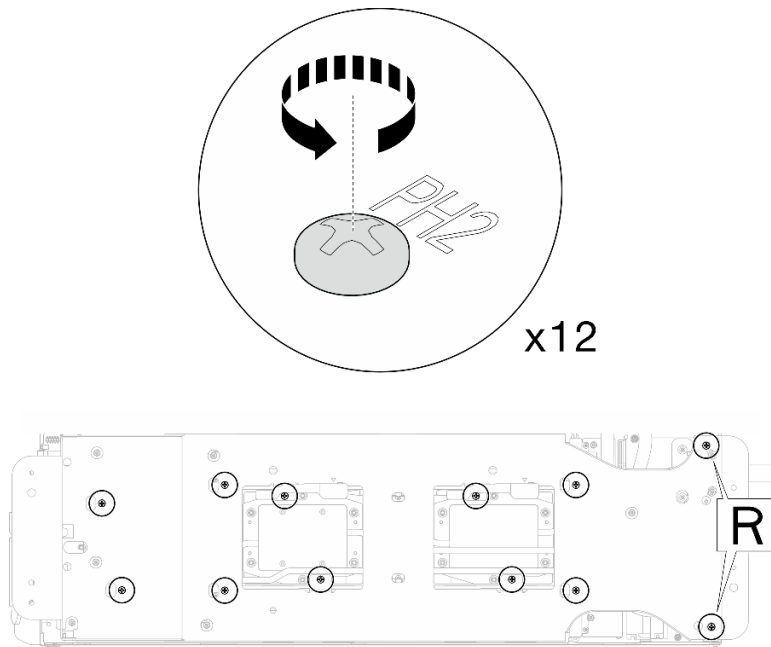
图 274. 拧松水循环模块载板的螺钉
