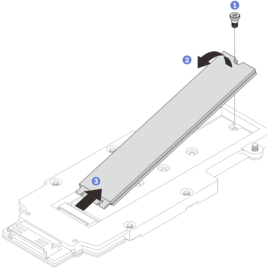
图 158. 卸下 M.2 硬盘
