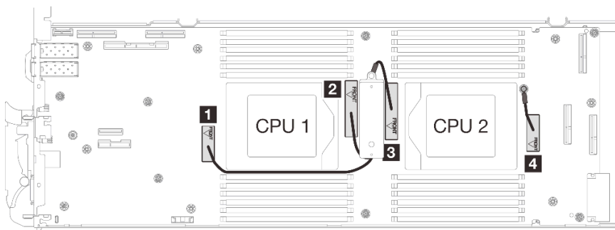
图 305. 屏蔽罩的线缆布放
