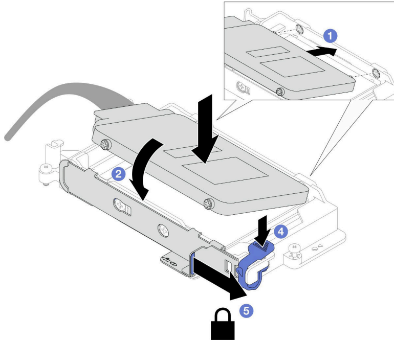
图 128. 安装上方硬盘
