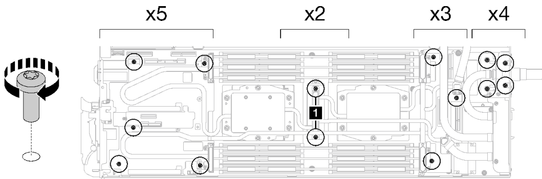
图 278. 安装水循环模块螺钉和快接件螺钉
