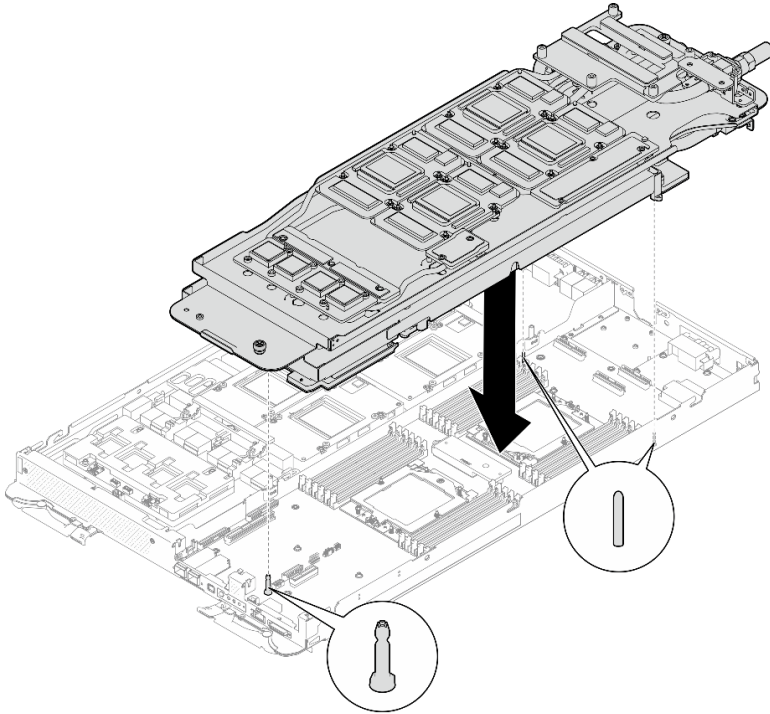
图 62. 安装水循环模块载板
