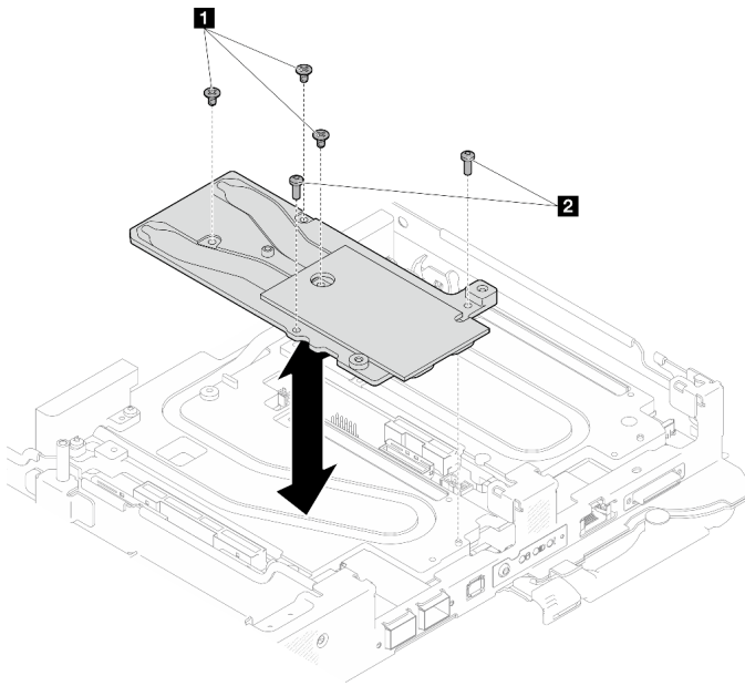
图 252. 安装 OSFP 模块导电板
