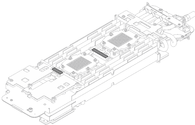
图 271. 水循环模块油灰垫
