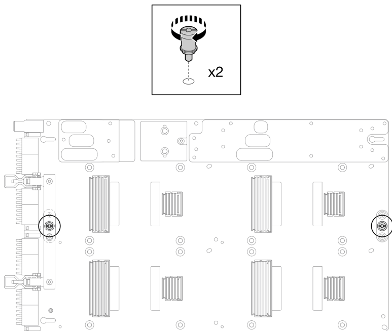
图 376. 将 T15 螺钉安装到 GPU 板上
