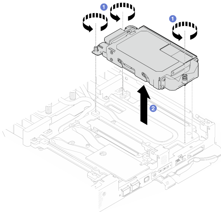
图 135. 卸下 E3.S 硬盘仓组合件
