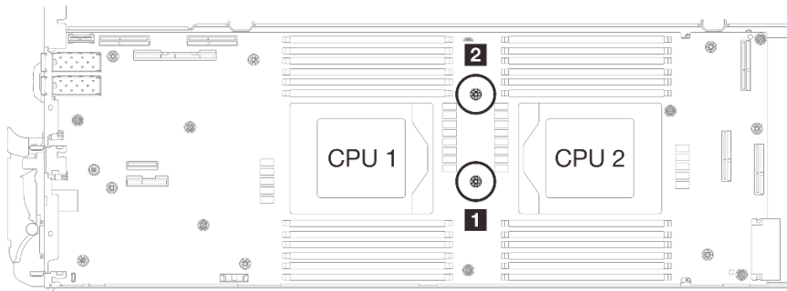
图 291. 屏蔽线缆 1/2 和 3 的螺钉孔的位置
