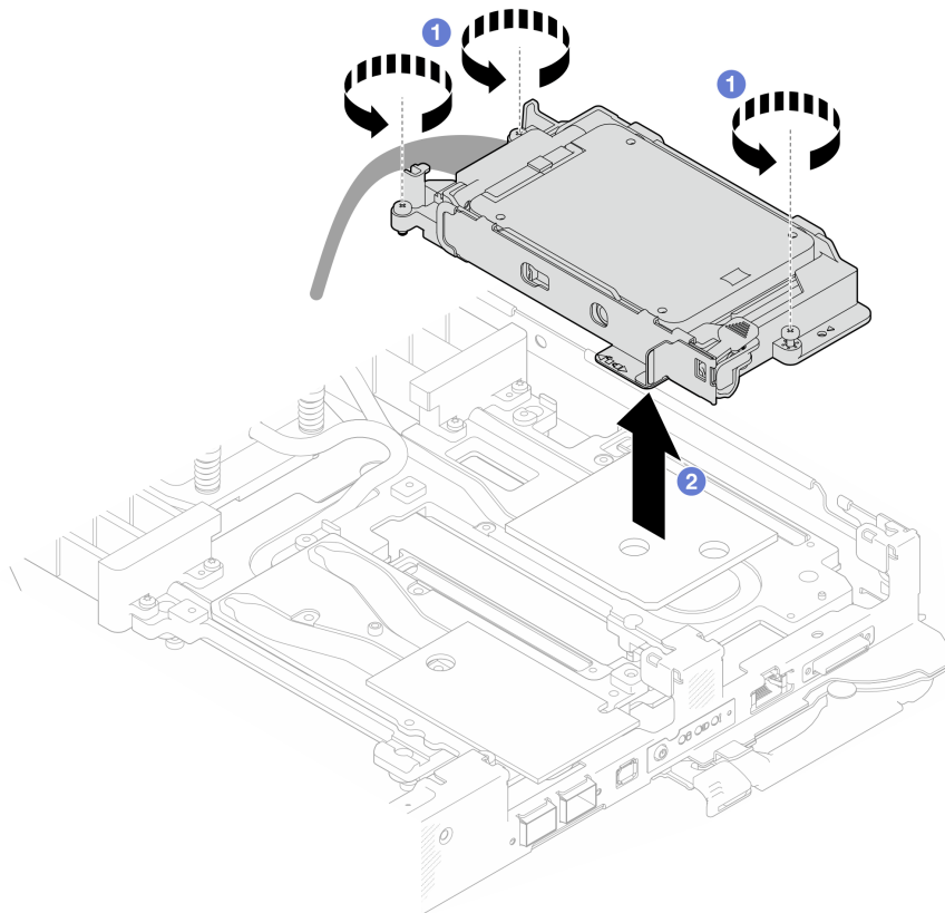
图 121. 卸下 7 毫米 NVMe 硬盘仓组合件
