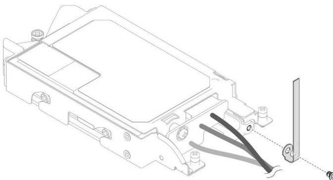
图 138. 取下线缆扎带
