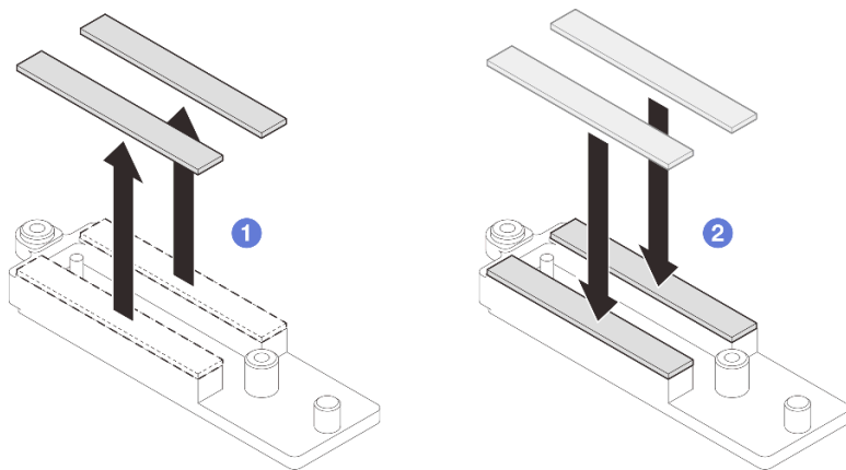
图 288. 更换 VR 导电板油灰垫
