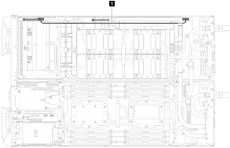
图 325. 拔下载板电源线
