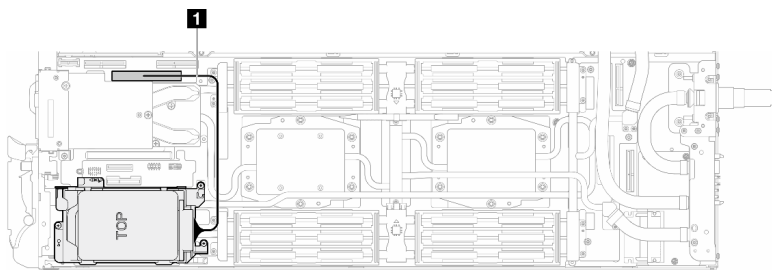
图 193. 连接硬盘线缆
