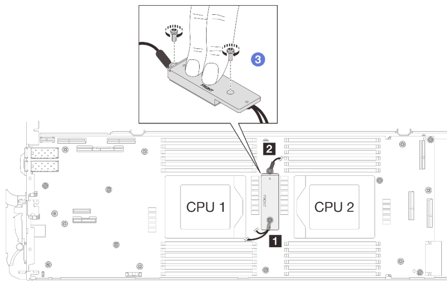
图 88. 连接屏蔽线缆 1/2 和 3
