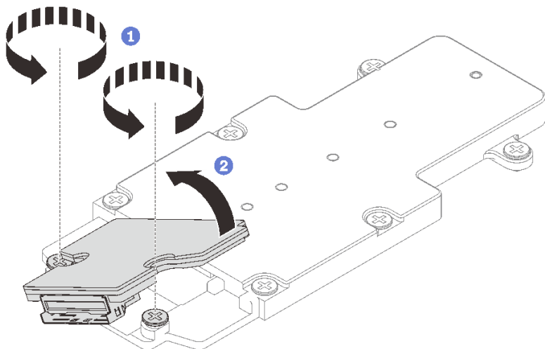
图 157. 拆卸 M.2 背板组合件
