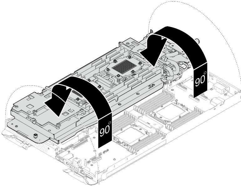
图 205. 折叠水循环模块
