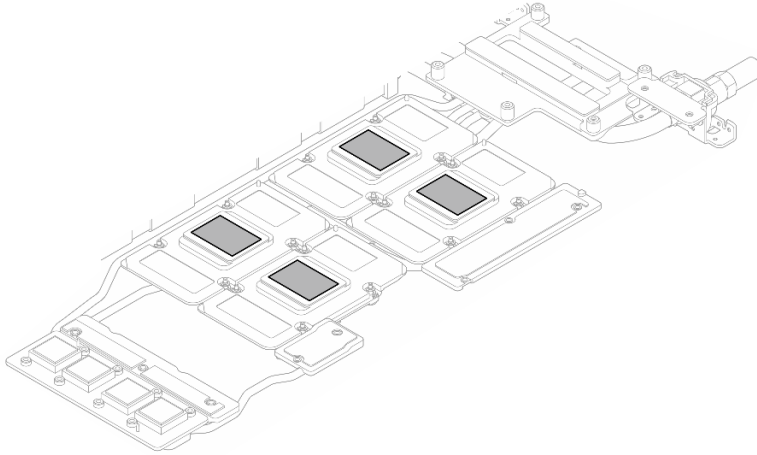
图 347. 清除所有 GPU 上的 PCM
