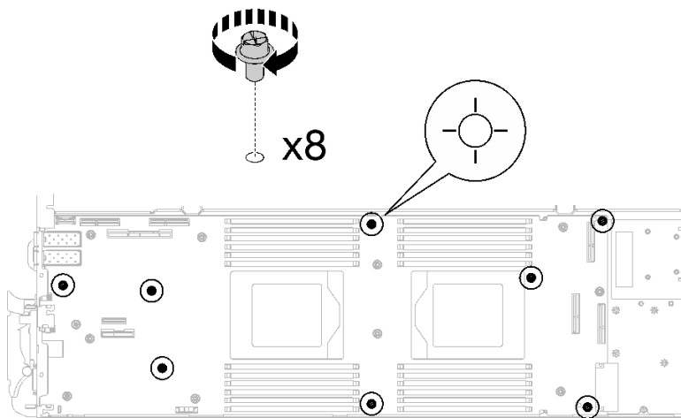
图 320. 安装主板螺钉
