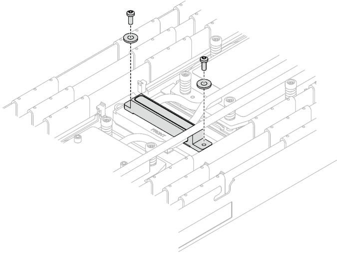
图 67. VR 冷却板螺钉以及垫圈
