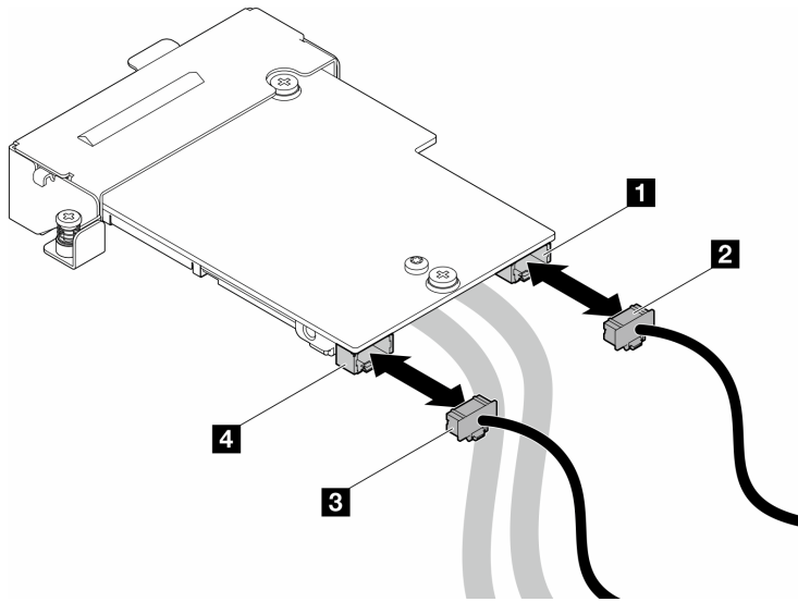
图 186. 拔下 OSFP 模块电源线
