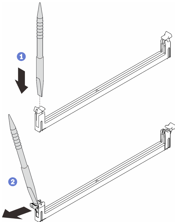
图 168. 卸下内存条
