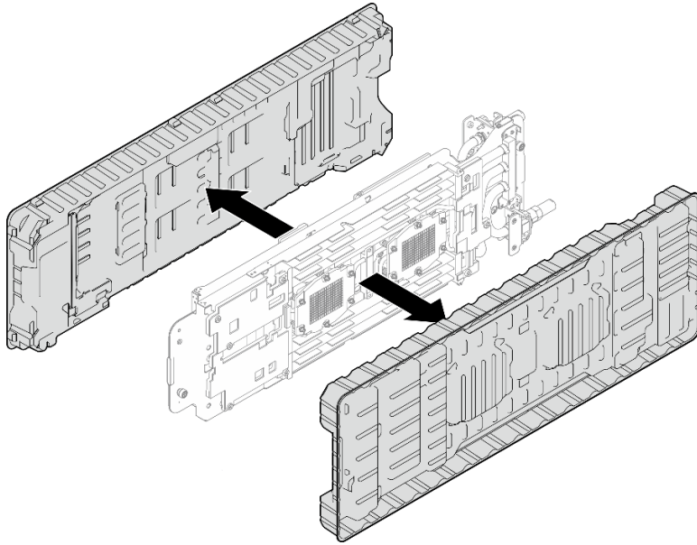
图 268. 卸下塑料油脂外盖
