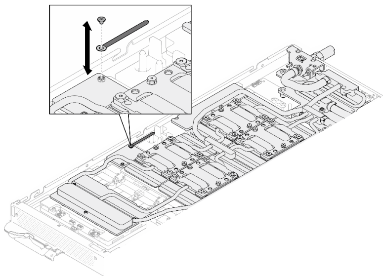
图 80. 安装线缆扎带
