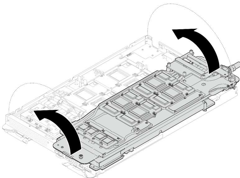
图 450. 将水循环模块展开到 GPU 节点上
