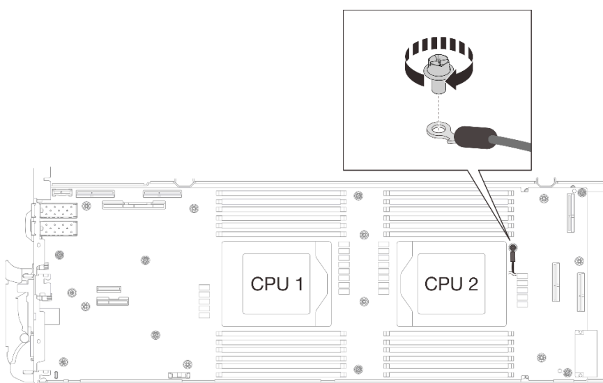
图 314. 连接屏蔽罩线缆 4
