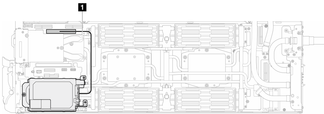
图 154. E3.S 硬盘线缆布放
