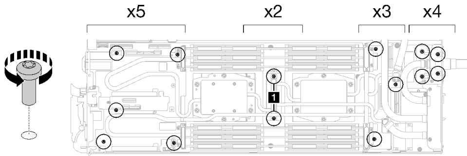
图 199. 卸下水循环模块螺钉
