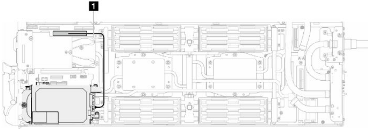
图 134. 拔下 E3.S 硬盘线缆
