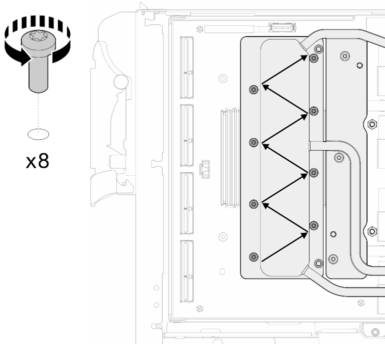
图 339. 卸下网卡螺钉
