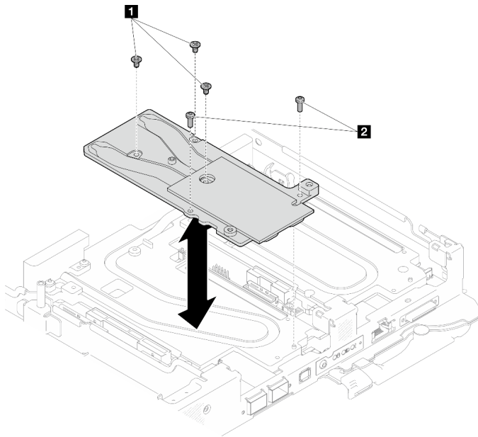
图 281. 安装 OSFP 模块导电板
