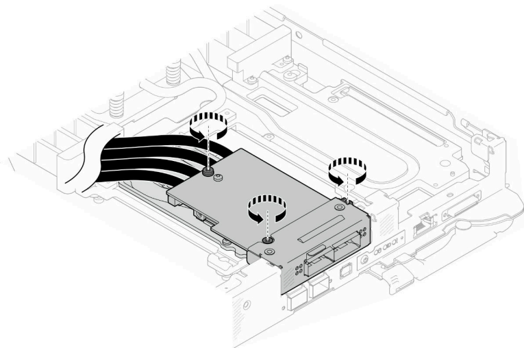
图 184. 卸下 OSFP 模块
