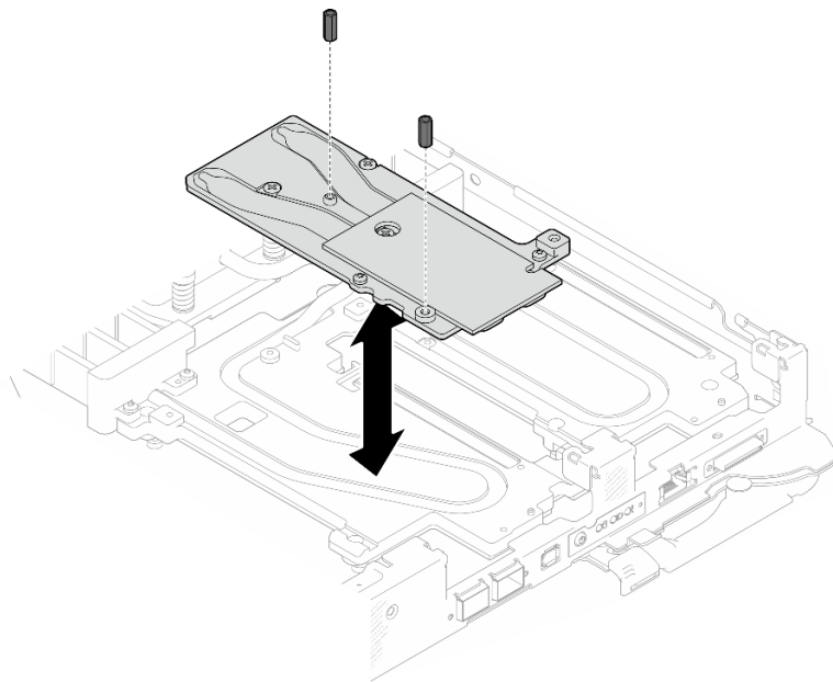
图 222. 安装 OSFP 模块导电板六角螺钉
