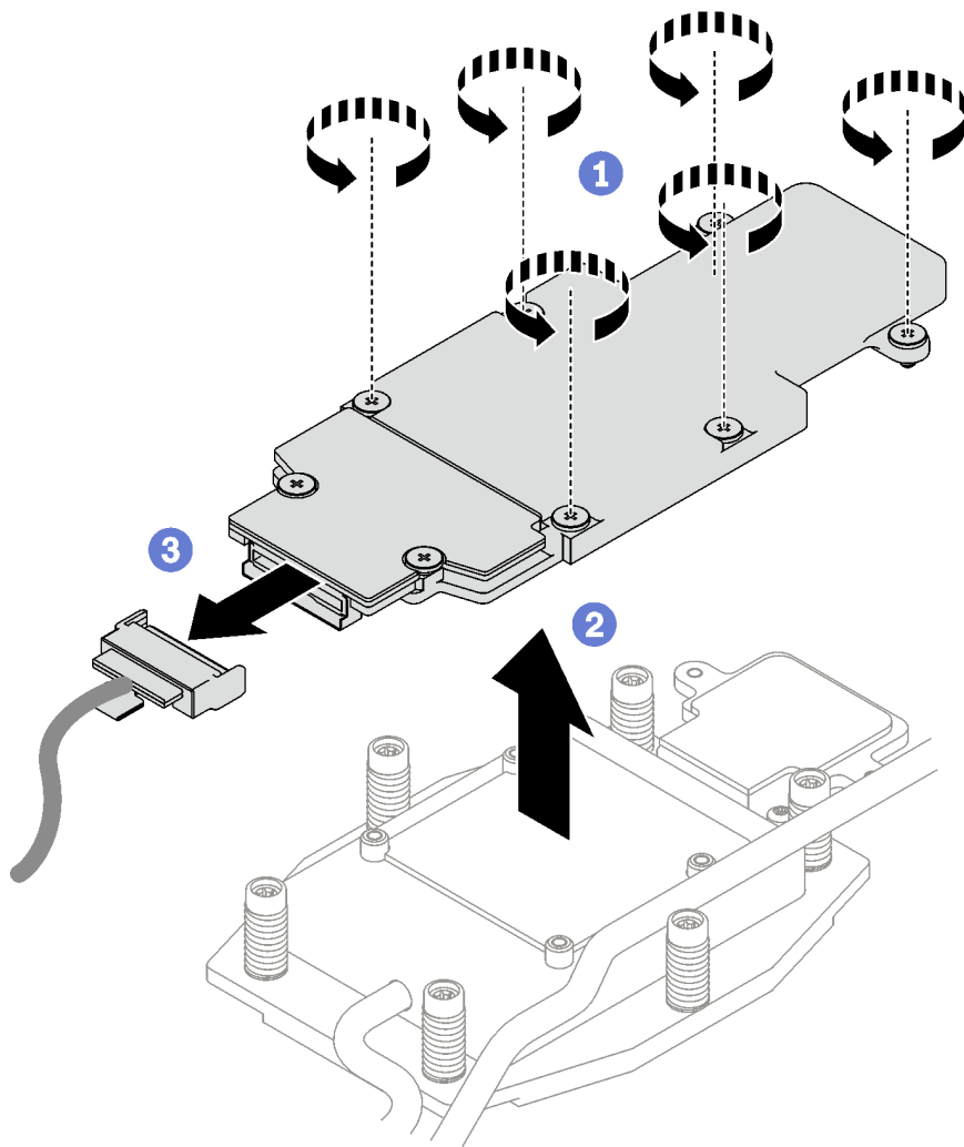
图 156. 卸下 M.2 背板组合件
