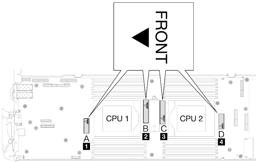
图 302. 屏蔽罩上的 FRONT 标记指向正面
