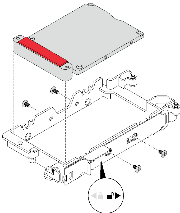
图 107. 卸下导电板
