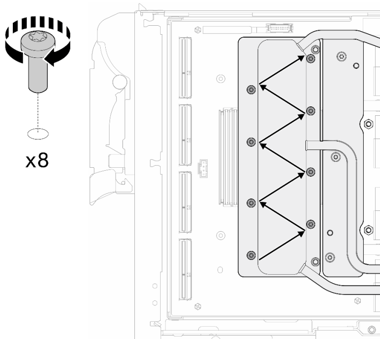
图 360. 安装网卡螺钉
