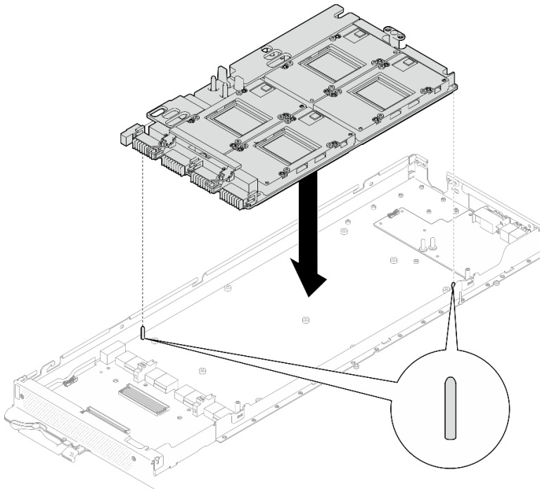
图 387. 将 GPU 板组合件安装到节点
