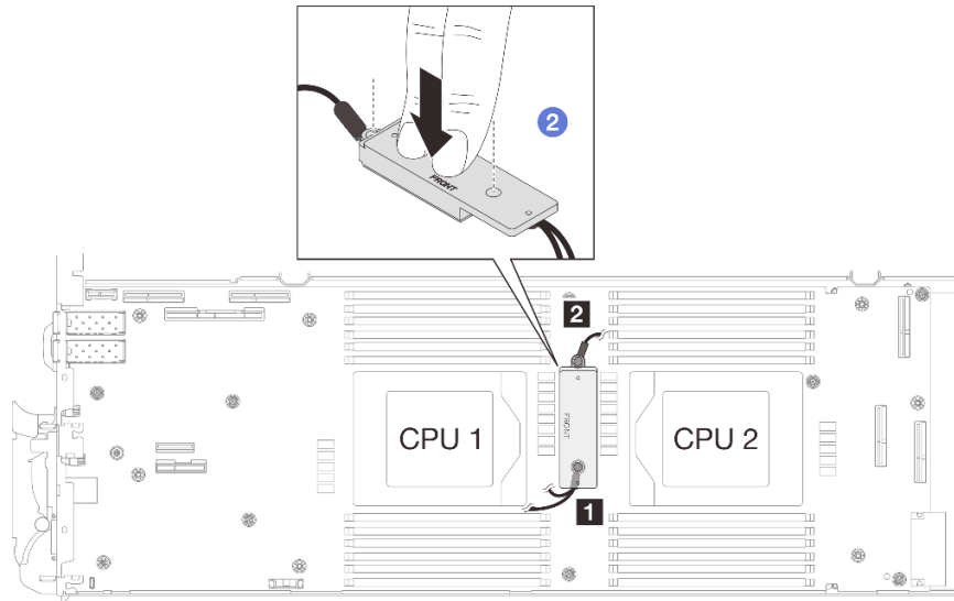
图 294. 按压 VR 导电板
