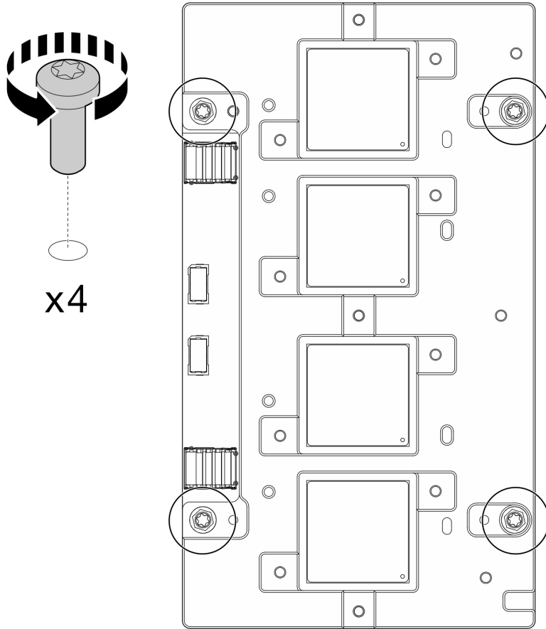
图 443. 卸下网卡螺钉
