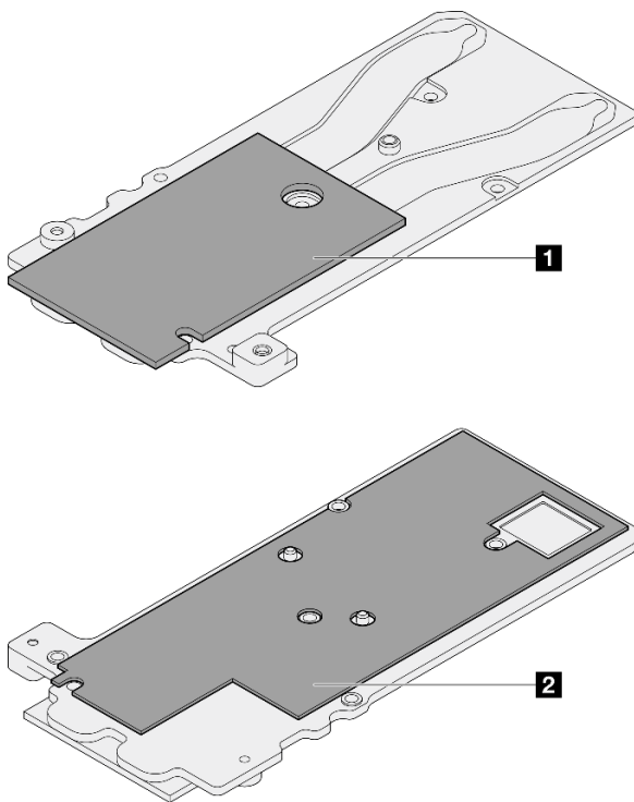
图 220. 更换 OSFP 模块导电板油灰垫
