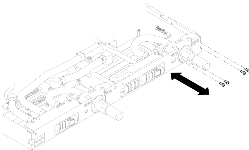
图 398. 卸下快接件螺钉 (GPU 节点)
