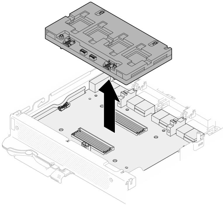
图 444. 卸下网卡
