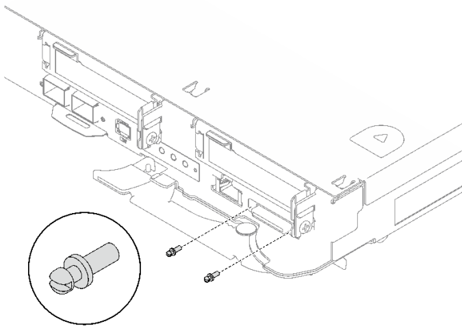
图 283. 卸下 KVM 螺钉
