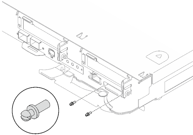
图 321. 安装 KVM 螺钉
