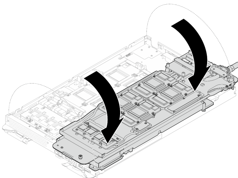
图 36. 将 GPU 节点侧水循环模块折叠到计算节点侧水循环模块上
