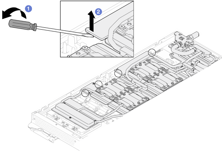
图 401. 从 GPU 板上松开正面和背面 MISC 导电板
