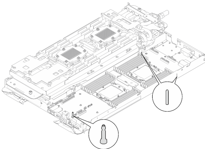
图 212. 计算节点上的导销
