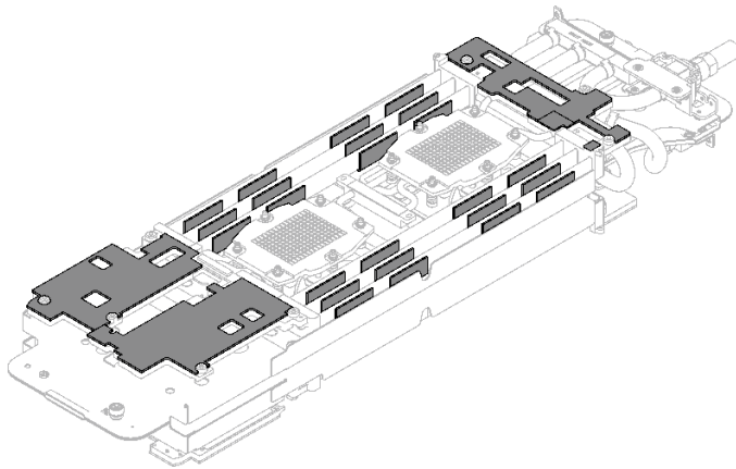
图 269. 水循环模块间隙垫（底面）
