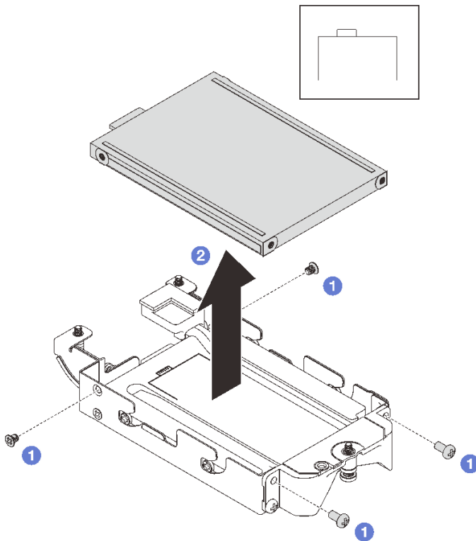
图 140. 卸下底部 E3.s 硬盘
