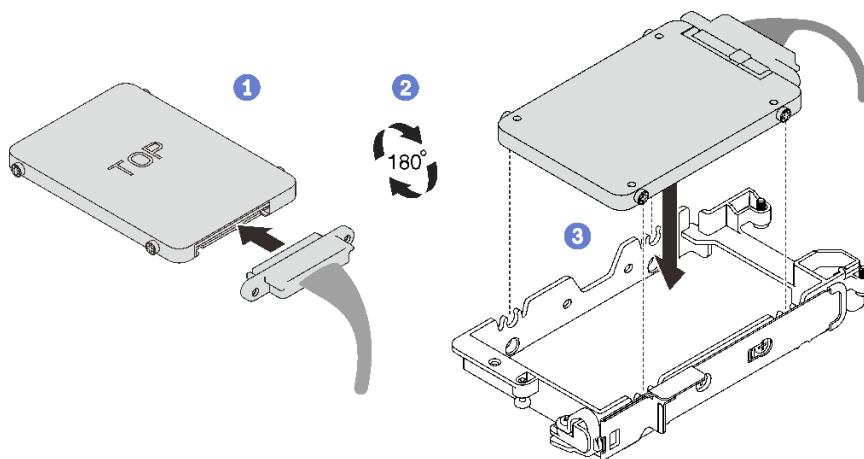
图 111. 安装下方硬盘 (7 毫米硬盘)
