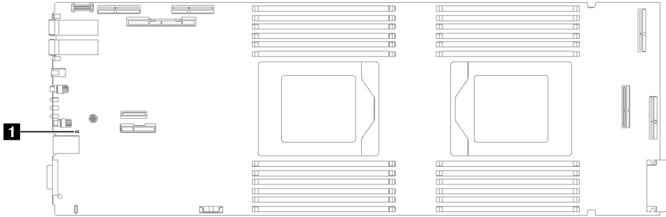
图 475. 主板 LED
