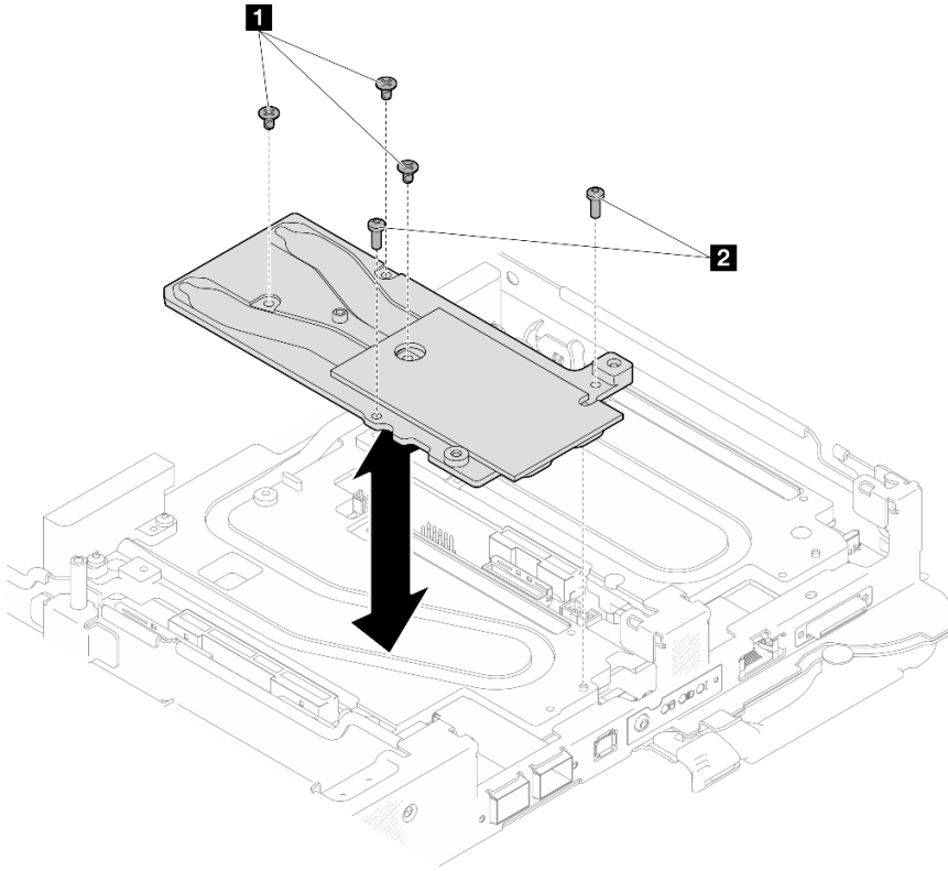
图 41. 卸下 OSFP 模块导电板
