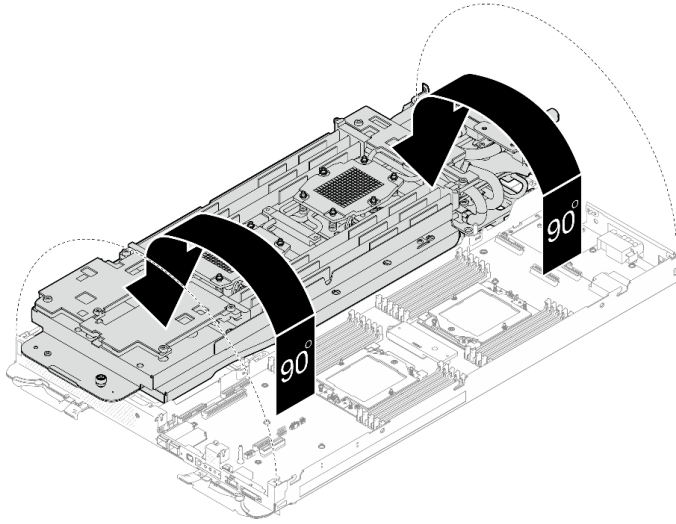
图 50. 折叠水循环模块
