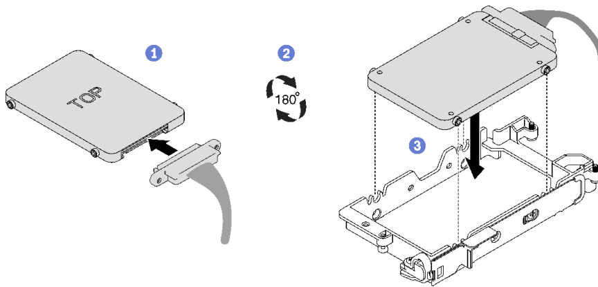
图 108. 安装 7 毫米硬盘
