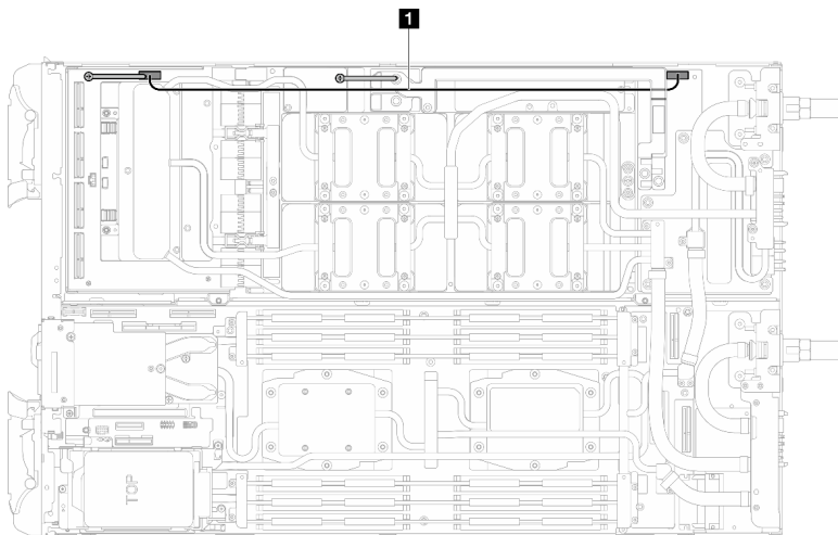
图 428. 拔下载板电源线
