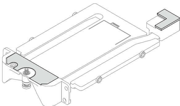
图 145. 更换导电板油灰垫
