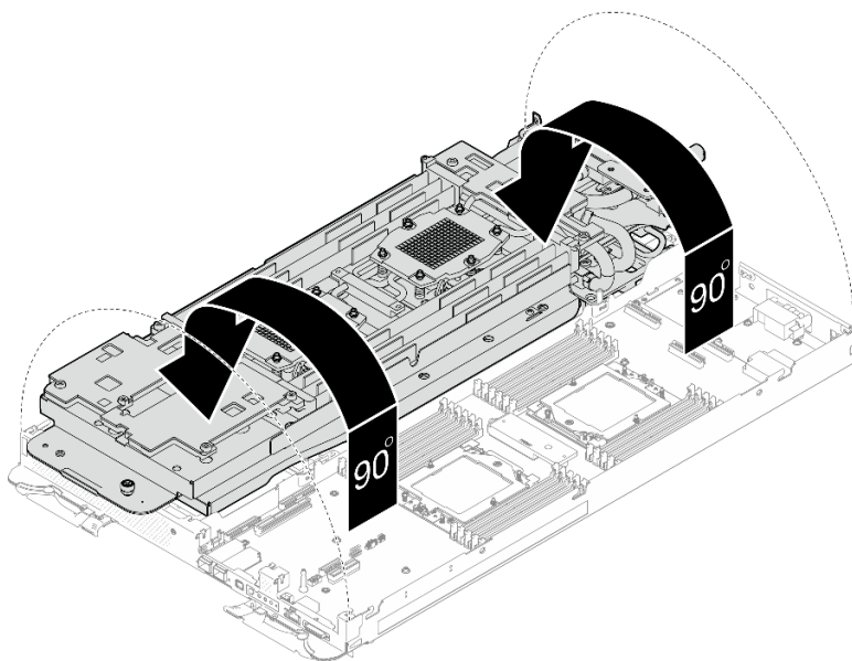
图 234. 折叠水循环模块
