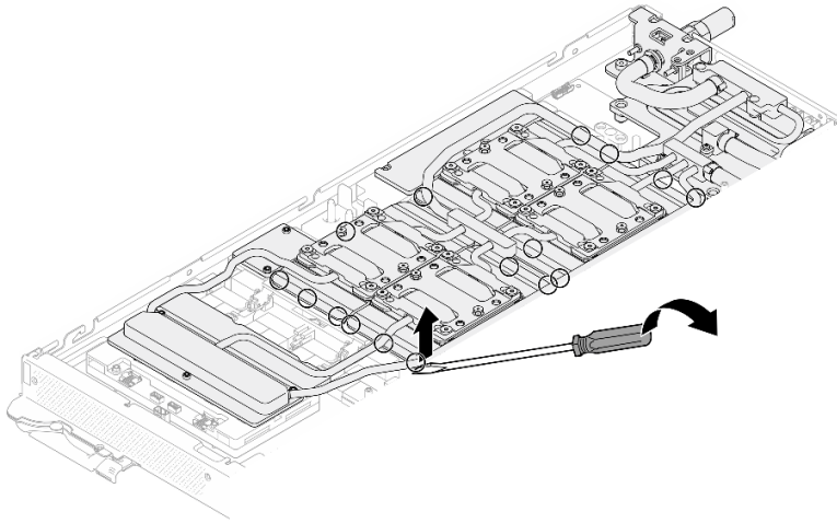
图 403. 从 GPU 上松开 GPU 冷却板
