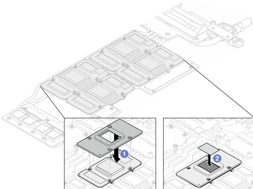
图 414. 更换水循环模块 GPU 冷却板 PCM (GPU 节点)
