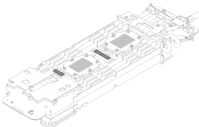
图 56. 水循环模块底面油灰垫（计算节点侧）
