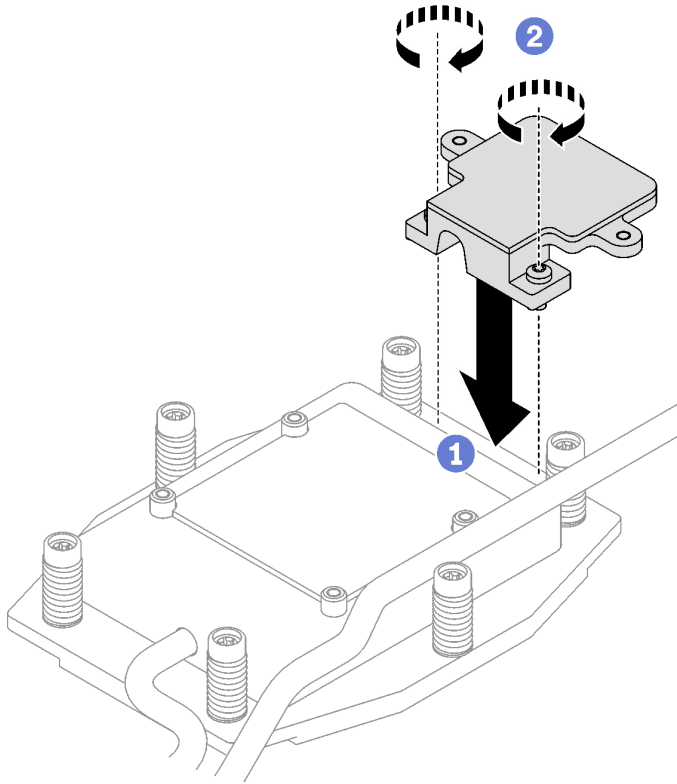
图 161. 安装 M.2 背板冷却板
