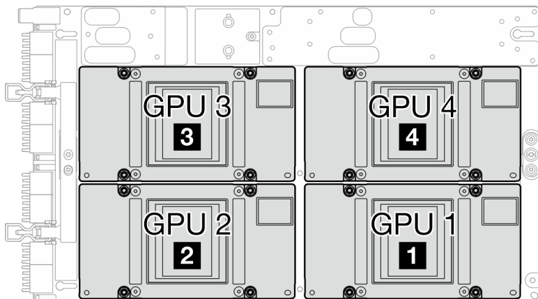
图 350. GPU 编号
