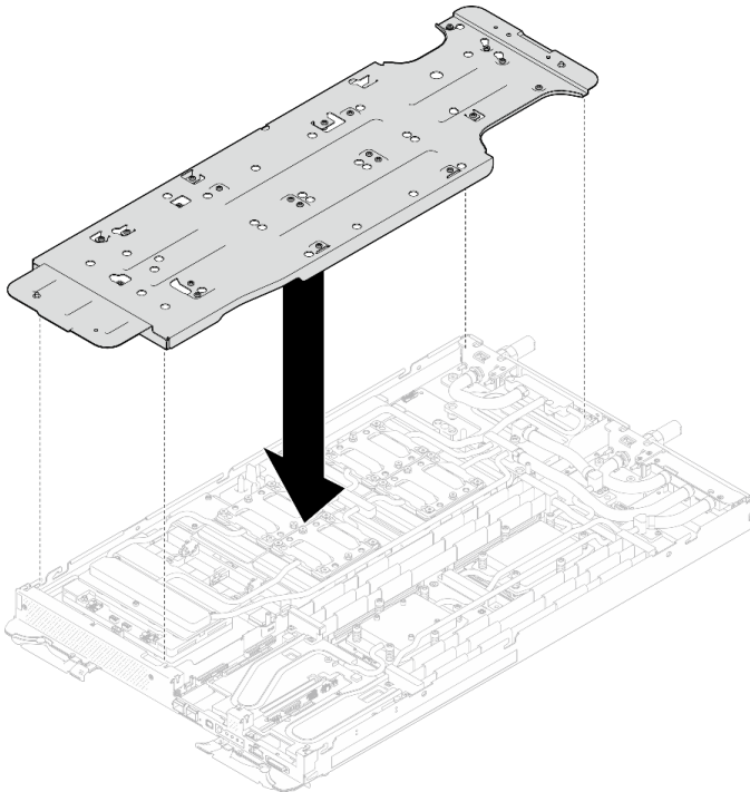
图 344. 安装水循环模块载板 (GPU 节点)
