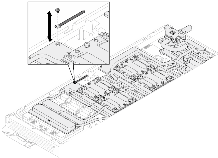
图 364. 安装线缆扎带
