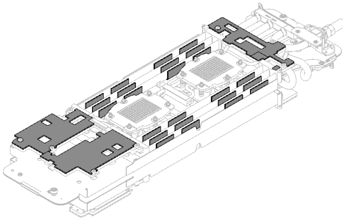
图 209. 水循环模块间隙垫（底面）
