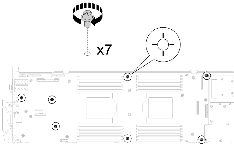
图 306. 安装主板螺钉
