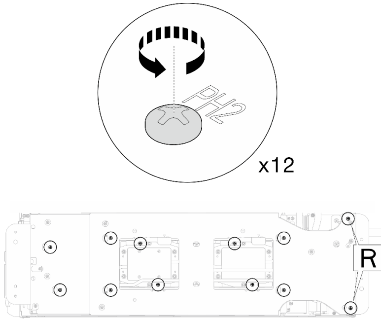
图 232. 安装水循环模块载板螺钉 (计算节点)
