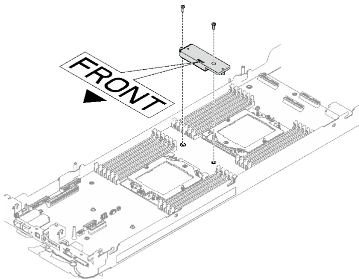
图 319. 安装 VR 导电板
