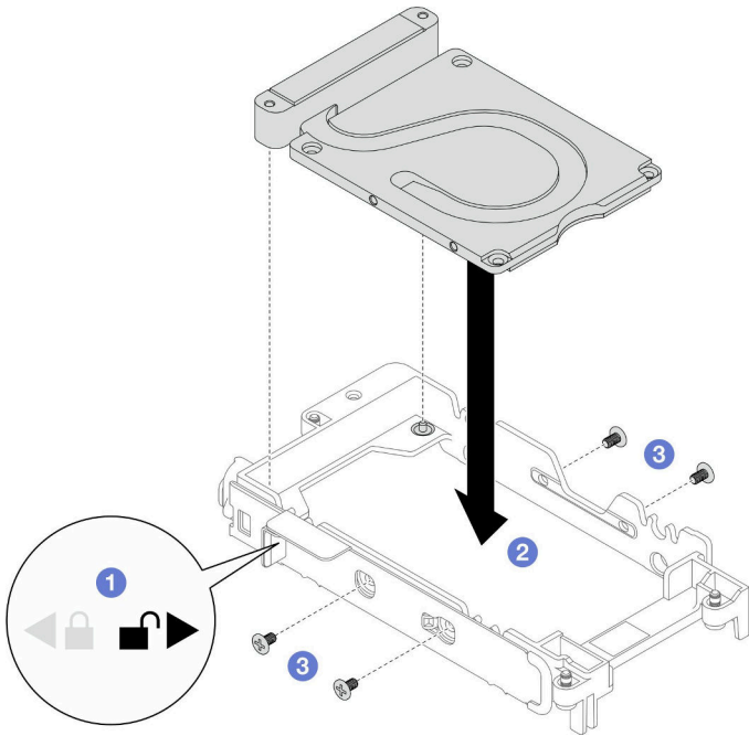
图 126. 安装导电板
