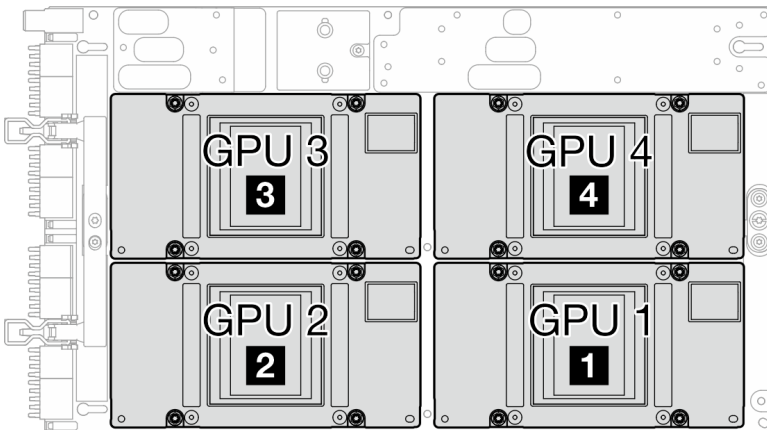
图 333. GPU 编号
