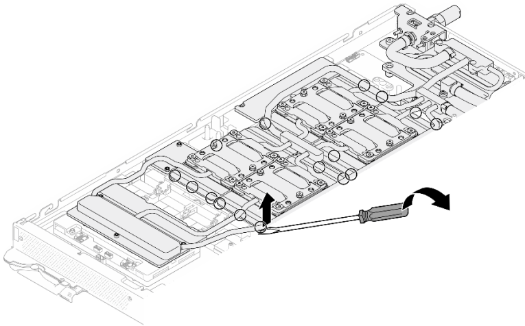
图 437. 从 GPU 上松开 GPU 冷却板
