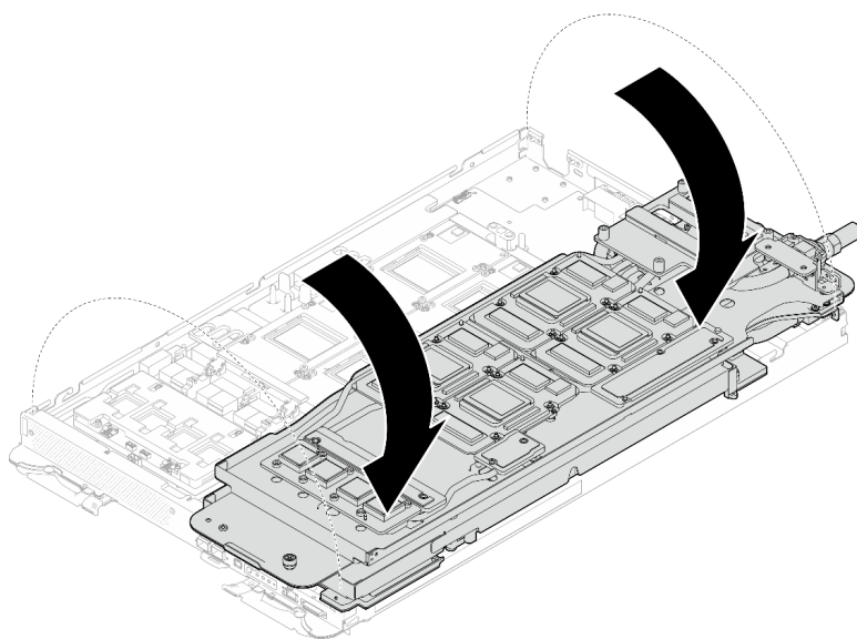
图 440. 将 GPU 节点侧水循环模块折叠到计算节点侧水循环模块上
