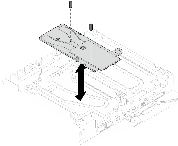
图 195. 卸下 OSFP 模块导电板六角螺钉
