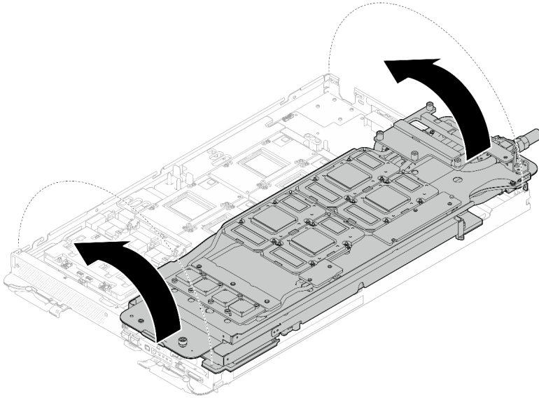
图 39. 将 GPU 节点水循环模块翻转回 GPU 节点中
