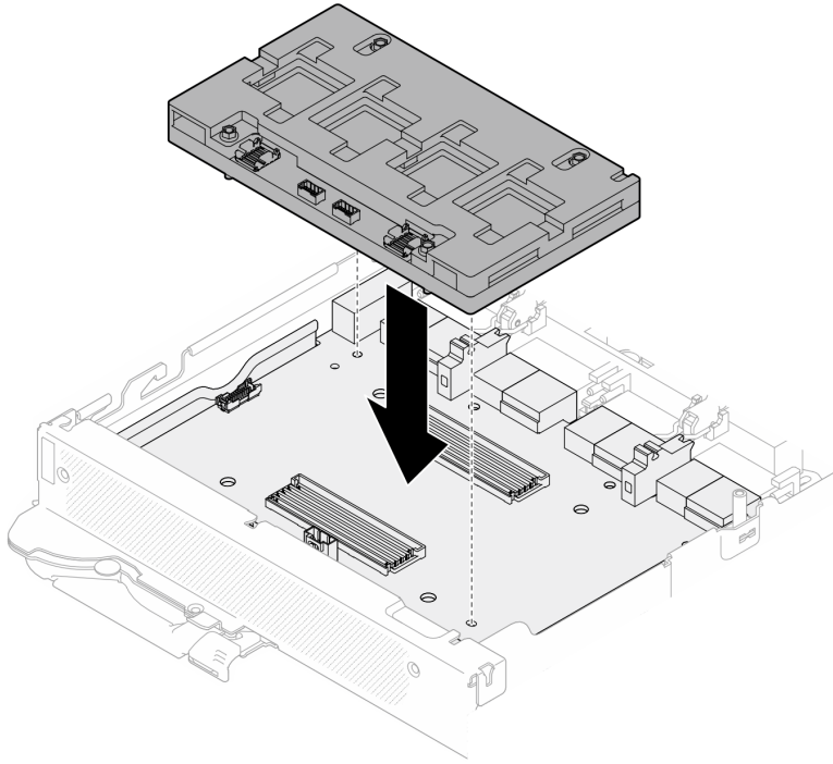
图 445. 安装网卡
