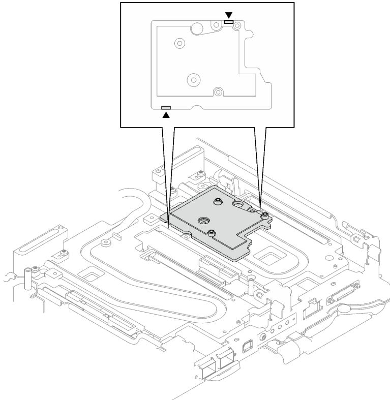
Abbildung 183. Positionen der Öffnungen an der Unterseite der Schnittstellenplatte
