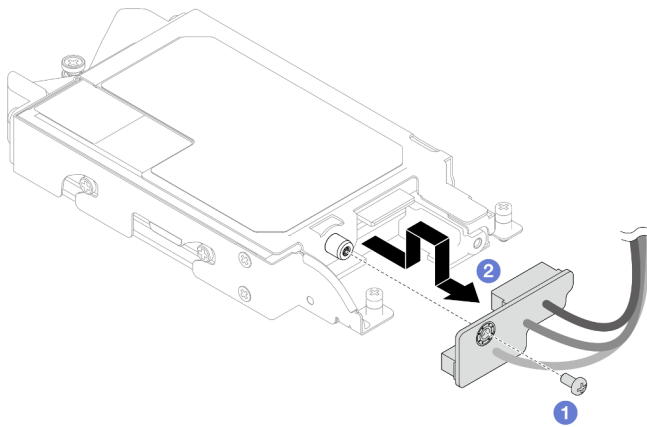
Abbildung 101. Entfernen der kabelgebundenen Rückwandplatine des E3.S-Laufwerks
