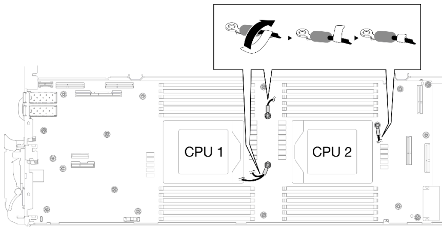
Abbildung 258. Rollen des Etiketts um das geschirmte Kabel
