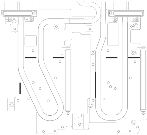
Abbildung 73. Markierungen auf dem Wasserkreislauf für die Ausrichtung des Gap Pad
