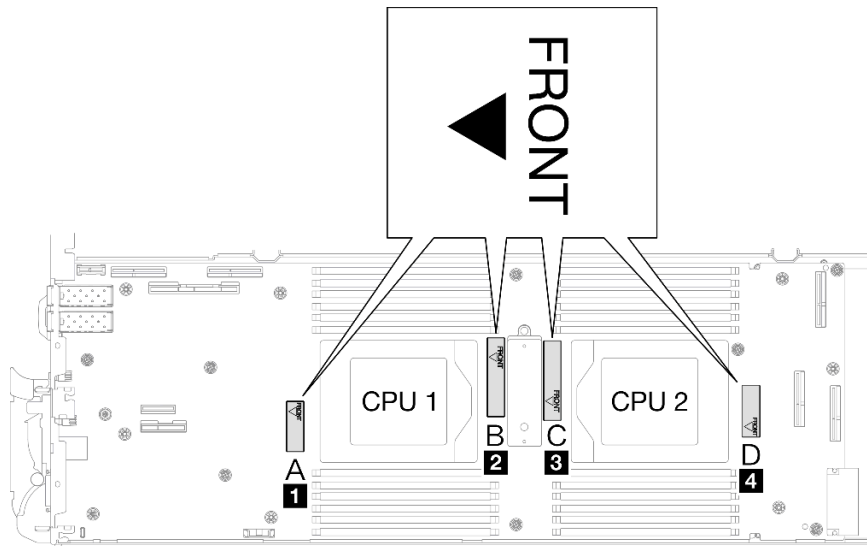
Abbildung 262. FRONT-Markierung auf dem Rahmen zeigt zur Vorderseite
