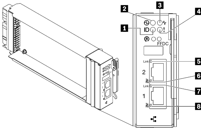
Abbildung 289. SMM2-Anzeigen
