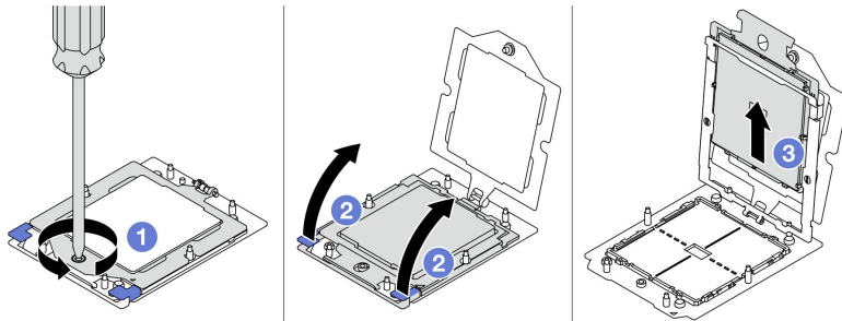
Abbildung 227. Entfernen eines Prozessors
