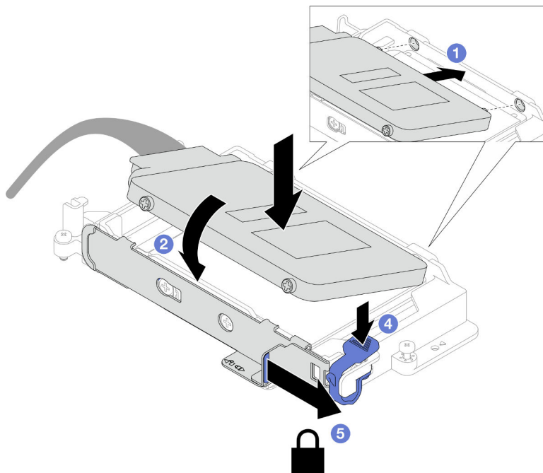
Abbildung 89. Installation des oberen Laufwerks
