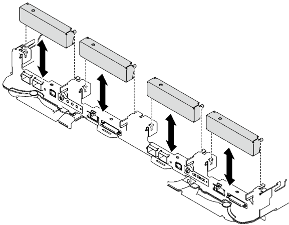
Abbildung 189. Entfernen der Abdeckblende für Frontblende
