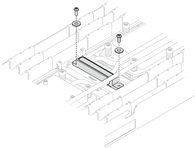
Abbildung 195. Schrauben der VR-Kühlplatte mit Unterlegscheiben
