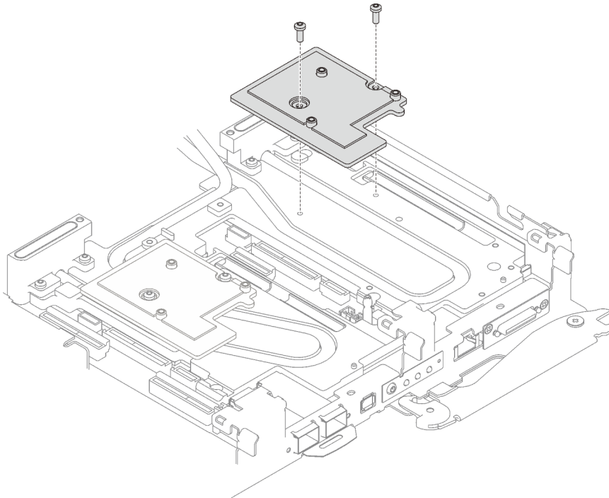
Abbildung 190. Installation der Schnittstellenplatte
