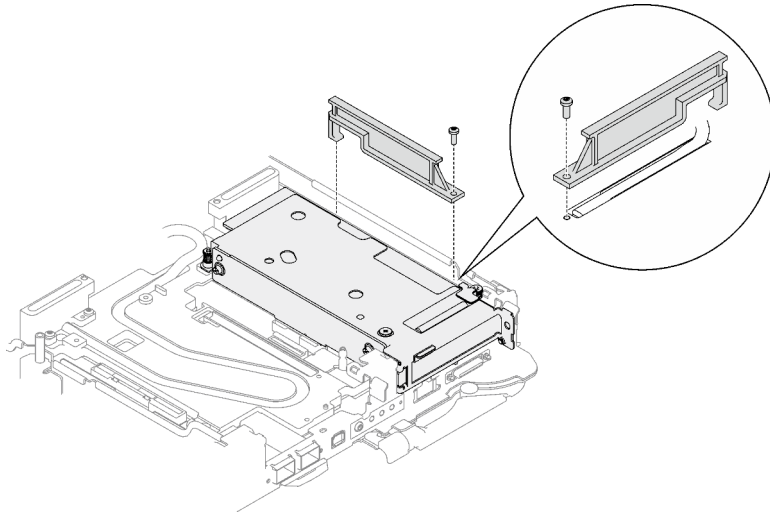
Abbildung 161. Installation des Wärmerohrträgers
