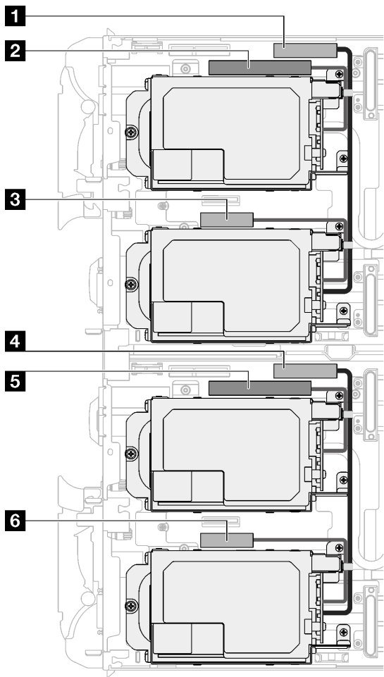
Abbildung 96. Verlegung des E3.s-Laufwerk-kabels
