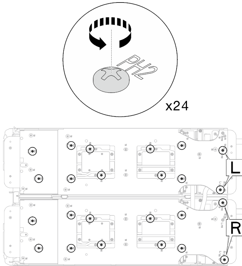
Abbildung 31. Lösen der Schrauben der Wasserkreislaufhalterung
