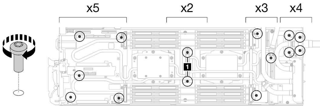
Abbildung 215. Installieren der Schrauben am Wasserkreislauf und Schnellanschluss
