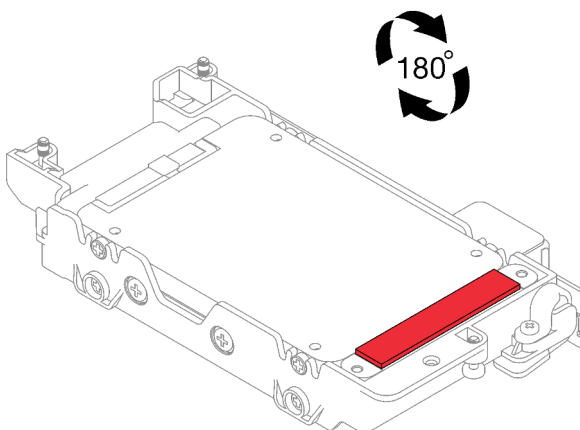
Abbildung 72. Position des Gap-Pads
