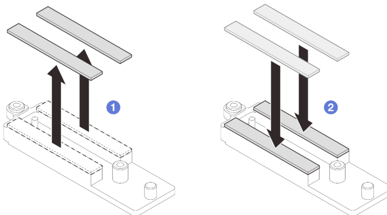
Abbildung 268. Austauschen der VR-Putty-Pads der Leiterplatte
