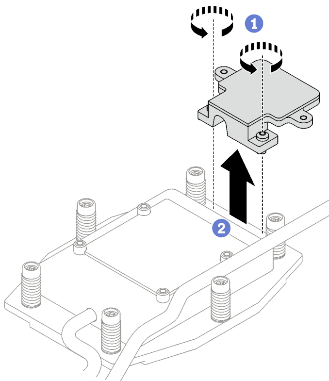
Abbildung 120. Entfernen der Kühlplatte der M.2-Rückwandplatine
