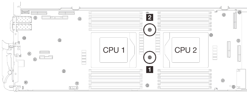
Abbildung 251. Position der Schraubenlöcher von geschirmtem Kabel 1/2 und 3
