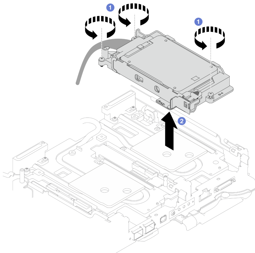
Abbildung 82. Entfernen der 7-mm-NVMe-Laufwerkhalterungsbaugruppe
