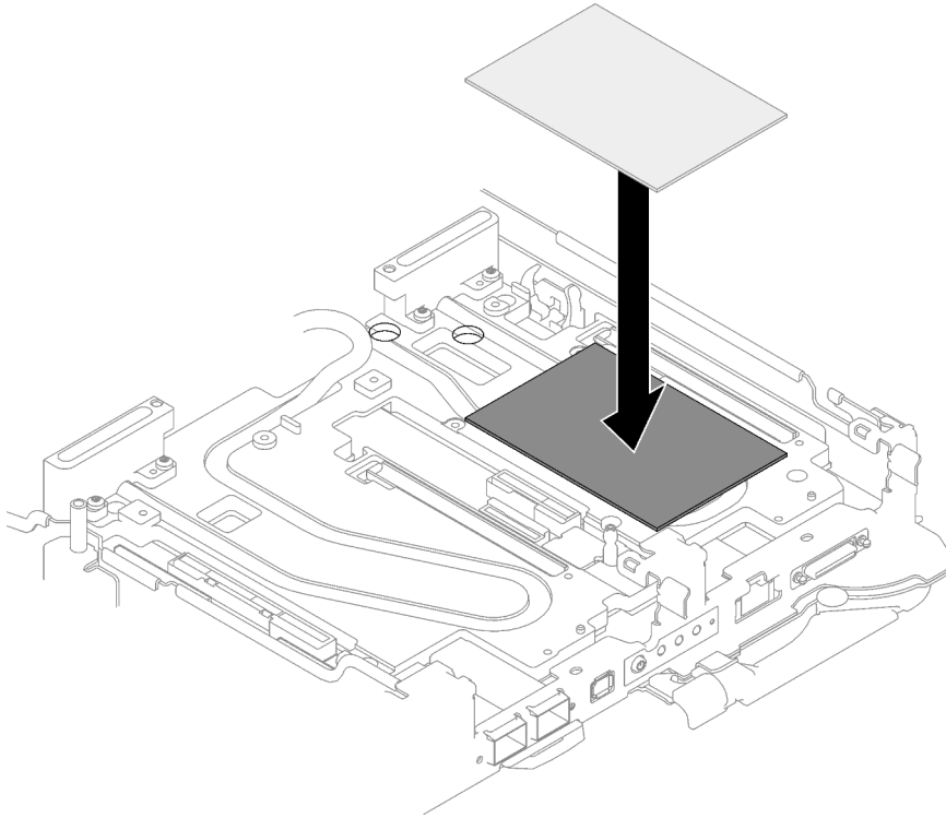
Abbildung 115. Austausch des Gap-Pads
