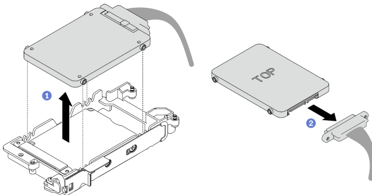
Abbildung 60. Entfernen eines 7-mm-Laufwerks
