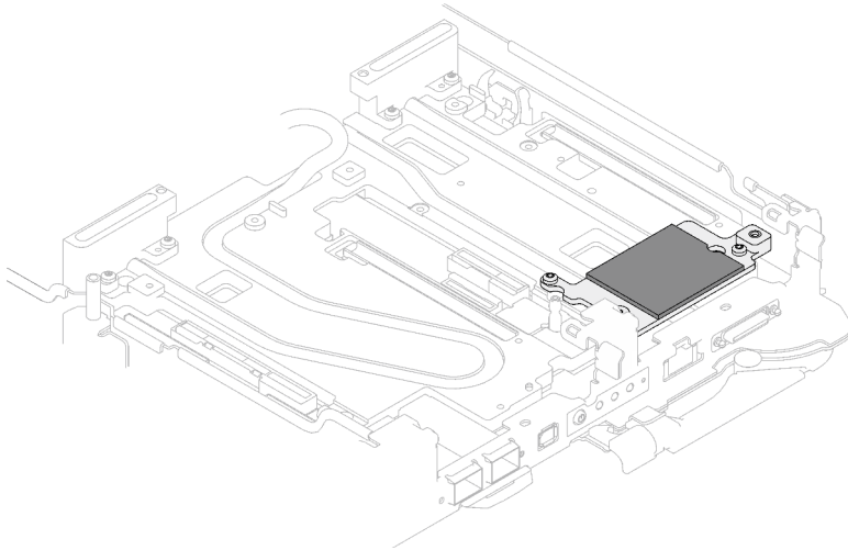
Abbildung 158. Schnittstellenplatten-Putty-Pad für CX-6 Adapterkarte
