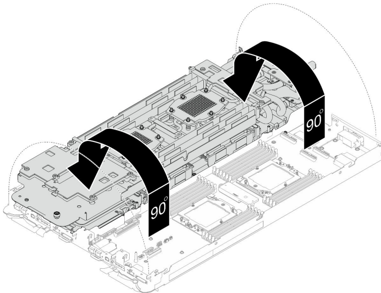
Abbildung 202. Wasserkreislauf falten
