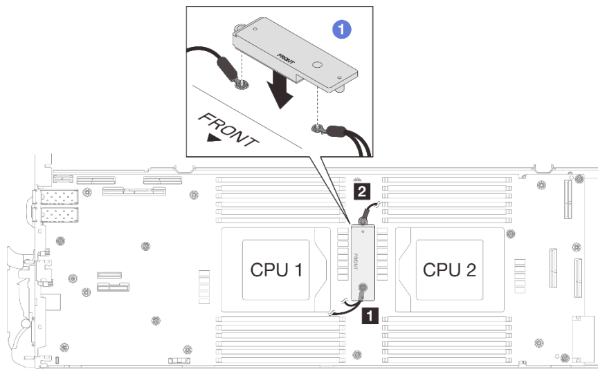
Abbildung 253. Ausrichten der VR-Leiterplatte, geschirmten Kabel und Schraubenlöcher auf der Systemplatine
