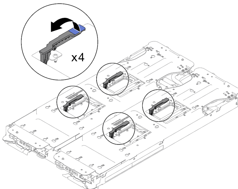
Abbildung 17. Trennen des Wasserkreislaufs vom Prozessor
