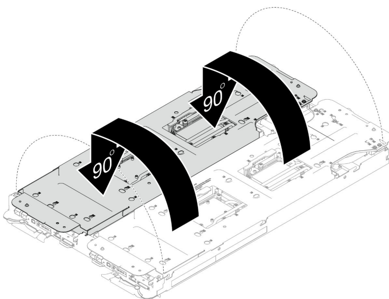
Abbildung 29. Aufklappen des Wasserkreislaufs
