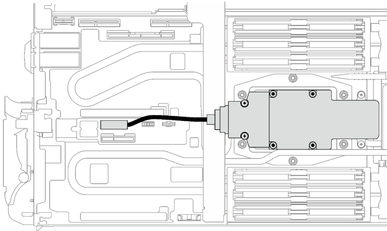
Abbildung 118. Entfernen des Kabels der M.2-Rückwandplattenbaugruppe
