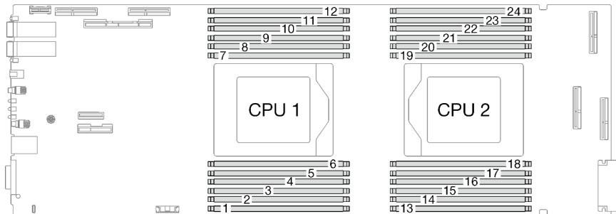
Abbildung 1. Layout für Speichermodule und Prozessoren
