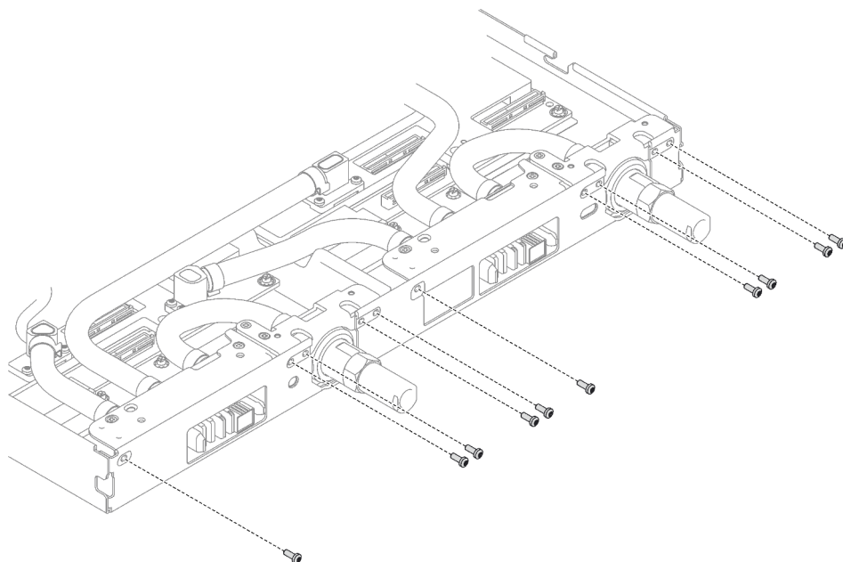
Abbildung 35. Installation der Schrauben am Schnellanschluss
