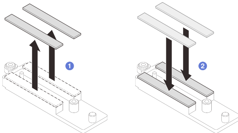
Abbildung 278. Austauschen der VR-Putty-Pads der Leiterplatte
