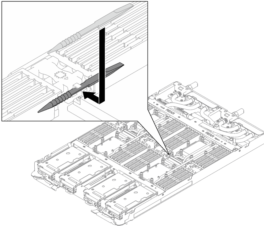
Abbildung 142. Befestigen des Speichermodul-Werkzeugs
