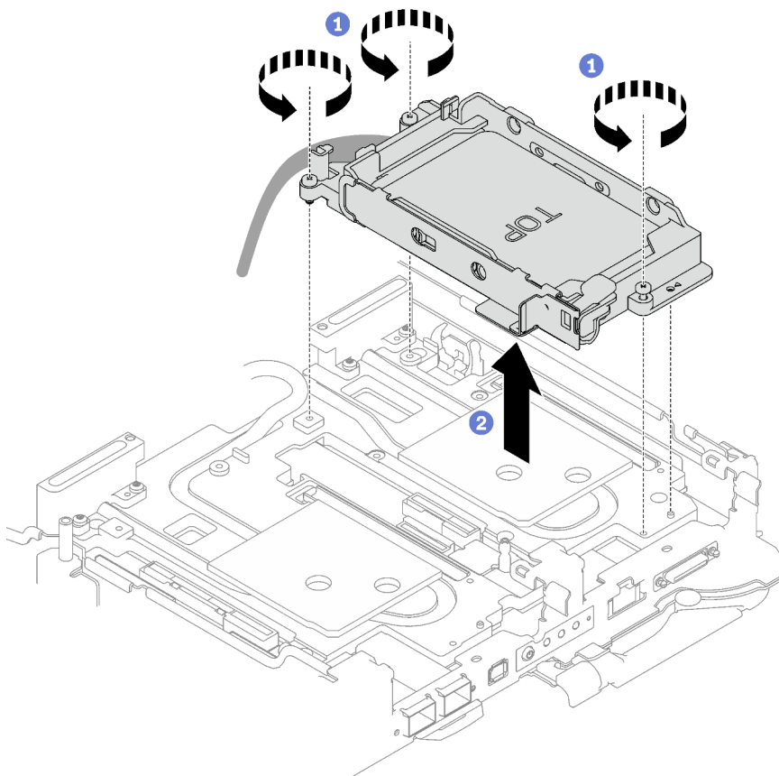
Abbildung 56. Entfernen der Laufwerkhalterung mit einem 7-mm-Laufwerk
