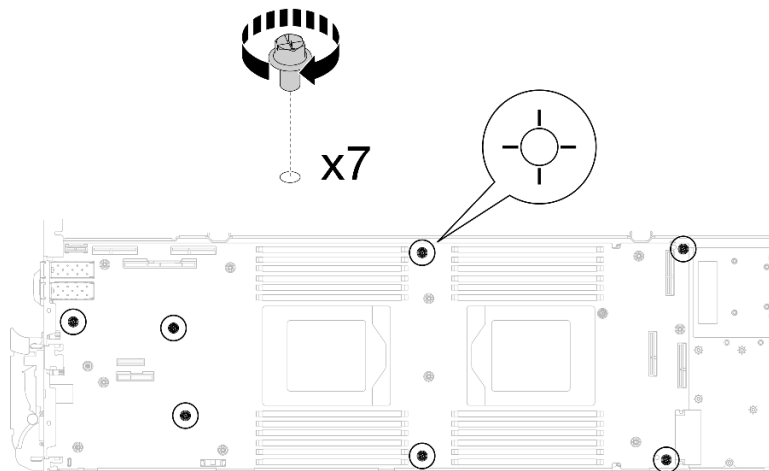
Abbildung 276. Anbringen der Systemplatinschrauben
