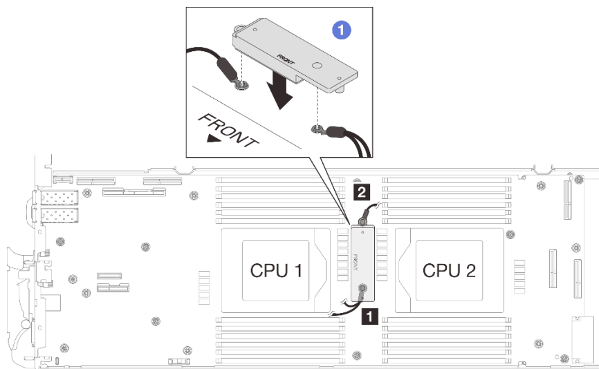
Abbildung 40. Ausrichten der VR-Leiterplatte, geschirmten Kabel und Schraubenlöcher auf der Systemplatine
