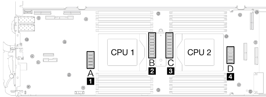
Abbildung 261. Positionen der Induktoren auf der Systemplatine
