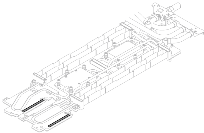
Abbildung 207. Gap-Pads am Wasserkreislauf (Oberseite)
