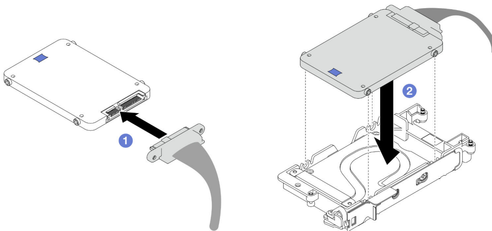
Abbildung 88. Installation des unteren Laufwerks
