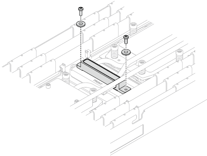
Abbildung 11. Schrauben der VR-Kühlplatte mit Unterlegscheiben
