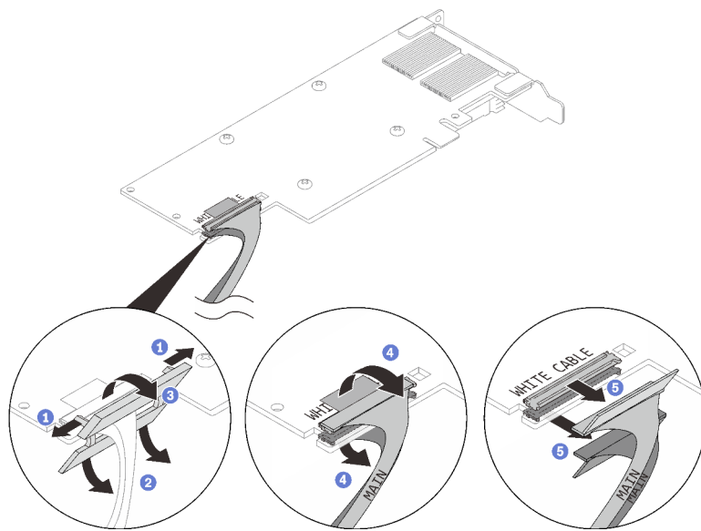
Abbildung 144. Entfernen des Kabels vom PCIe-Adapter
