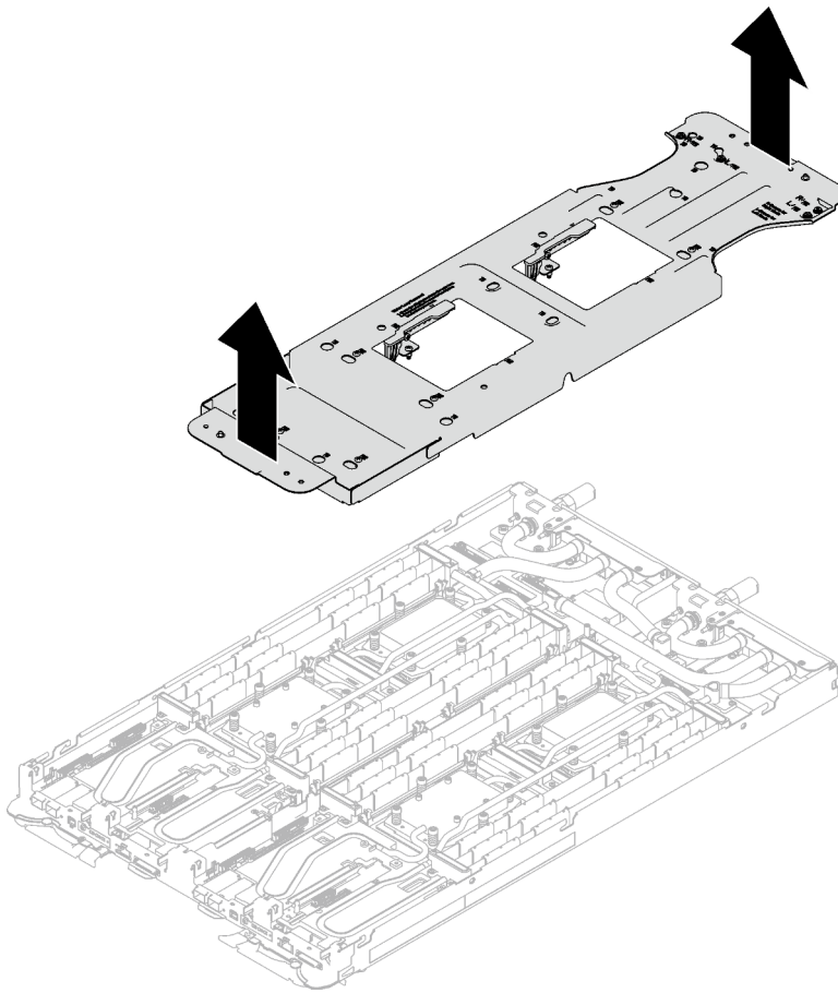
Abbildung 213. Wasserkreislaufhalterung entfernen
