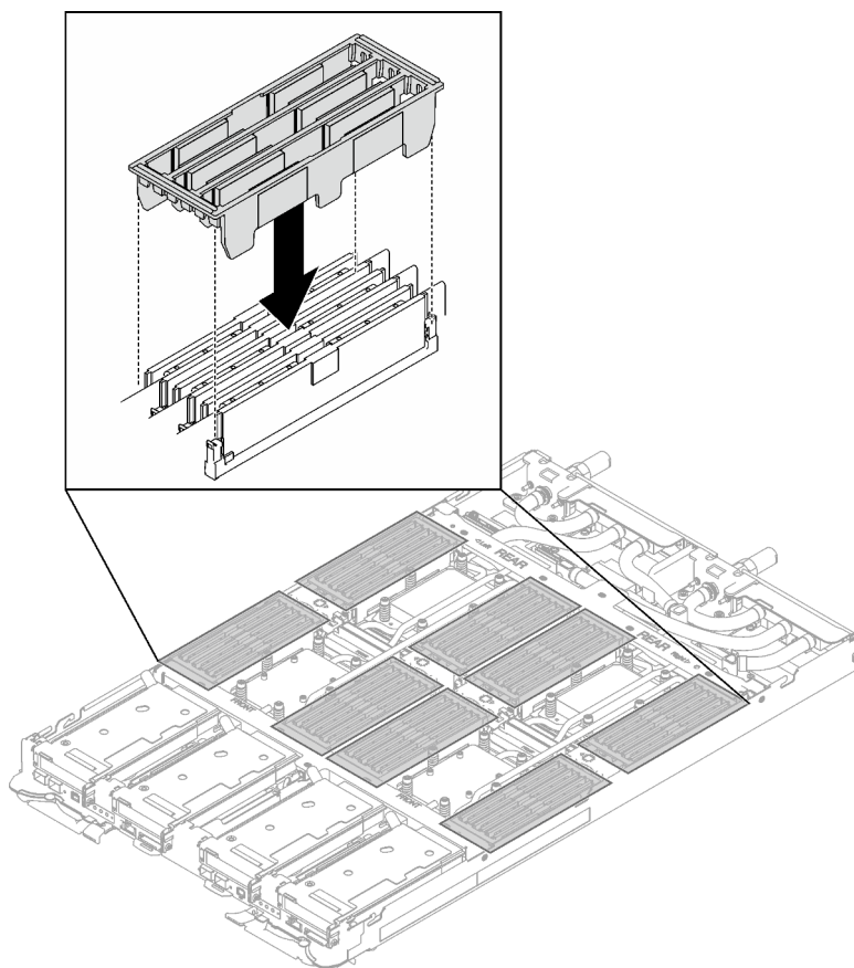
Abbildung 141. Installation der DIMM-Abdeckung
