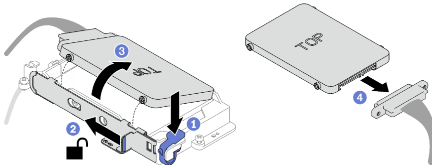
Abbildung 62. Entfernen des oberen Laufwerks
