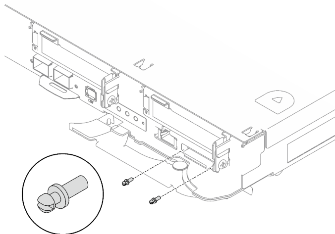
Abbildung 267. Anbringen der KVM-Schrauben
