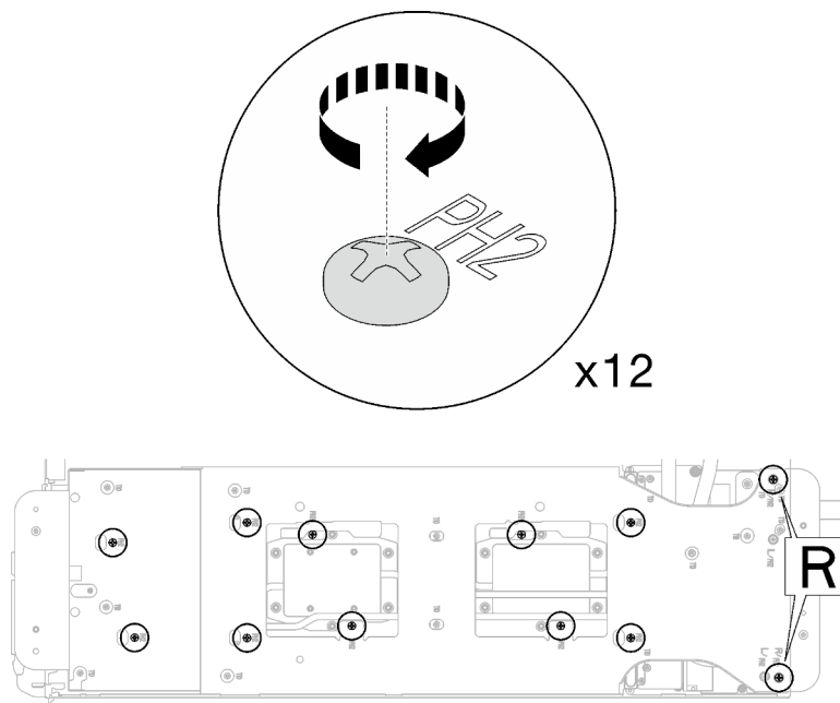
Abbildung 222. Installation der Schrauben der Wasserkreislaufhalterung
