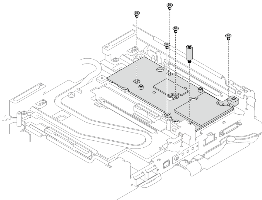
Abbildung 165. Entfernen der Schnittstellenplattenschrauben
