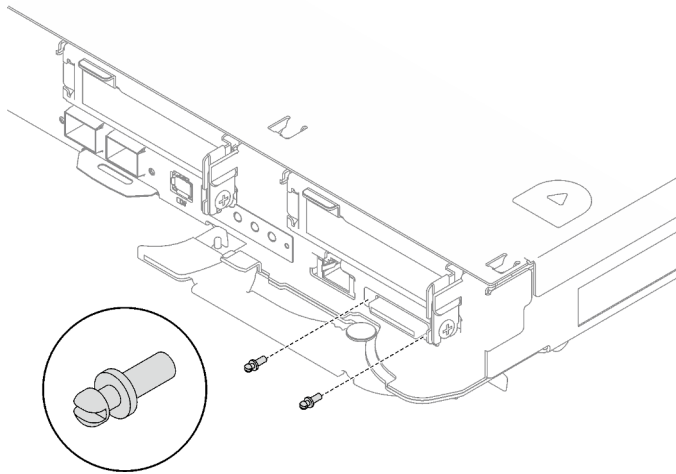
Abbildung 281. Anbringen der KVM-Schrauben
