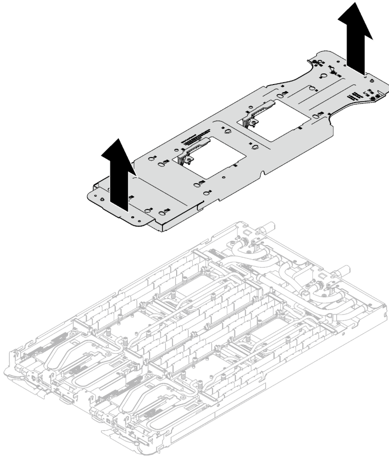
Abbildung 239. Wasserkreislaufhalterung entfernen
