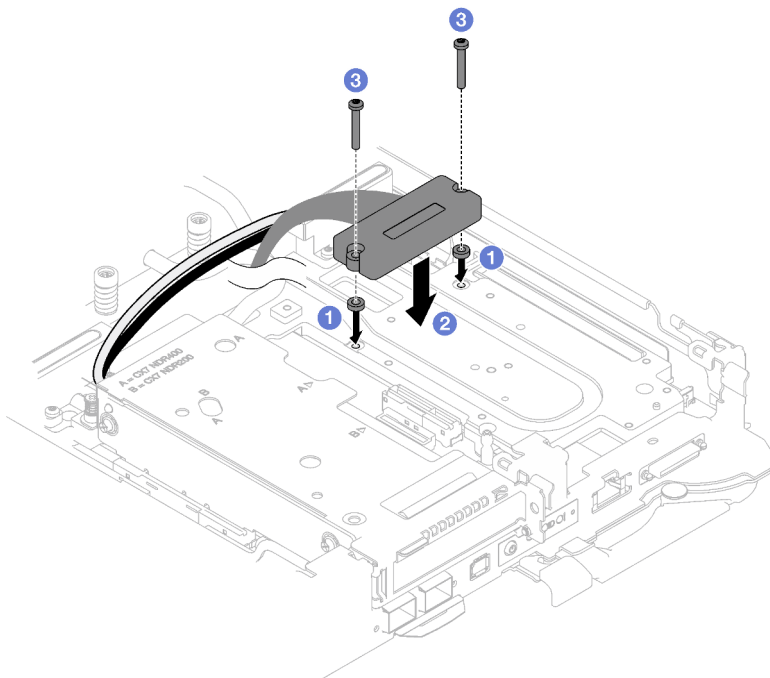
Abbildung 177. Verbindungskabel installieren
