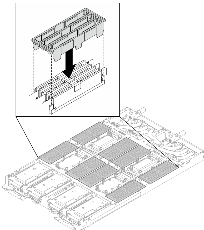
Abbildung 134. Installation der DIMM-Abdeckung
