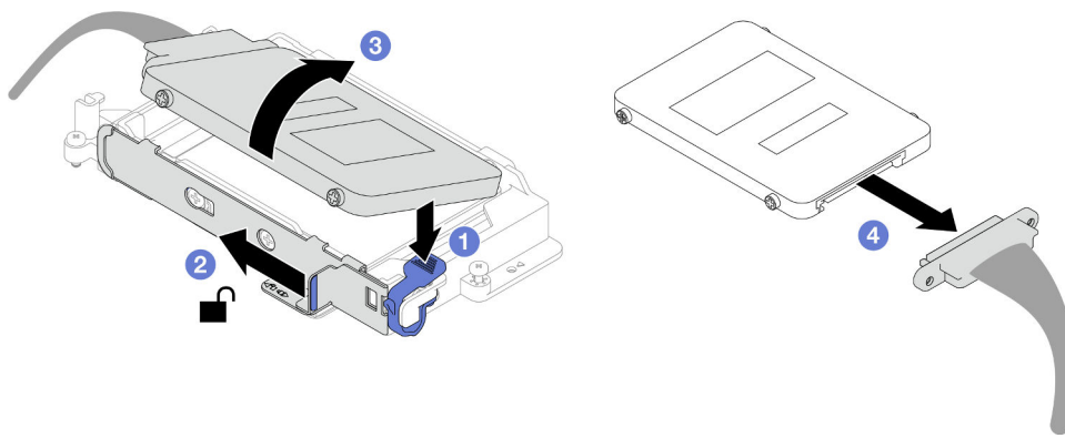
Abbildung 84. Entfernen des oberen Laufwerks (7-mm-NVMe)
