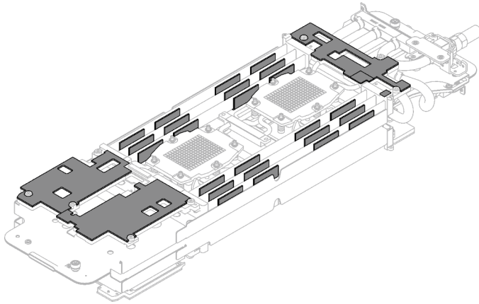
Abbildung 232. Gap-Pads am Wasserkreislauf (Unterseite)
