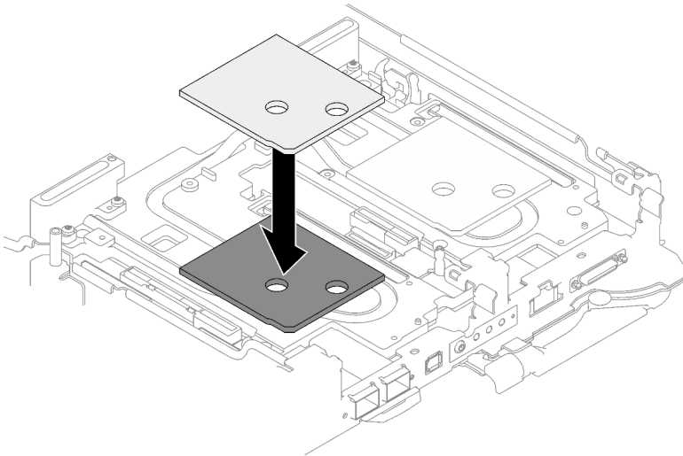
Abbildung 74. Austausch des Gap-Pads
