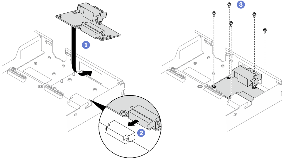
Abbildung 204. Installation der Stromversorgungsplatine
