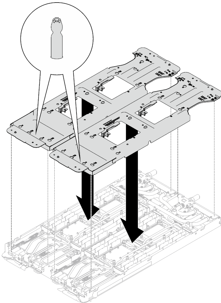
Abbildung 13. Installieren der Wasserkreislaufhalterung
