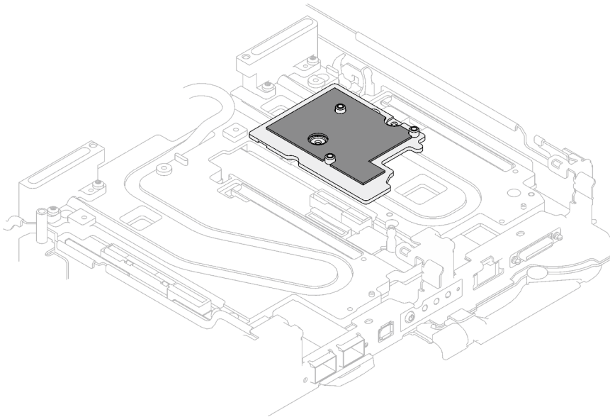
Abbildung 191. Gap-Pad auf Schnittstellenplatte für CX-7 NDR 400
