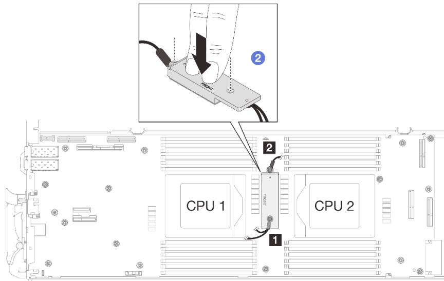
Abbildung 271. Drücken auf die VR-Leiterplatte
