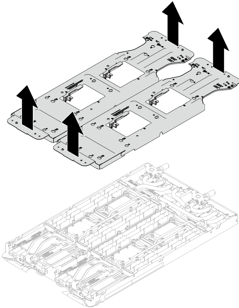
Abbildung 32. Wasserkreislaufhalterung entfernen
