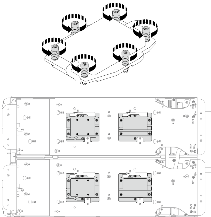
Abbildung 200. Entfernen der Prozessorkühlplatte
