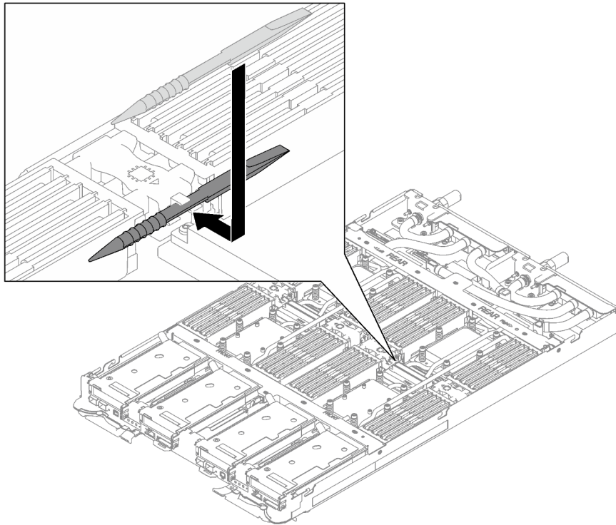
Abbildung 135. Befestigen des Speichermodul-Werkzeugs
