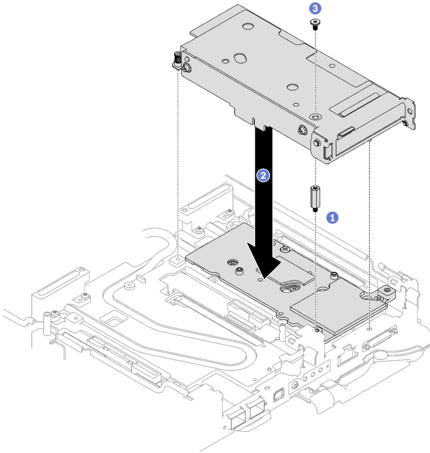
Abbildung 175. PCIe-Adapterkartenbaugruppe installieren
