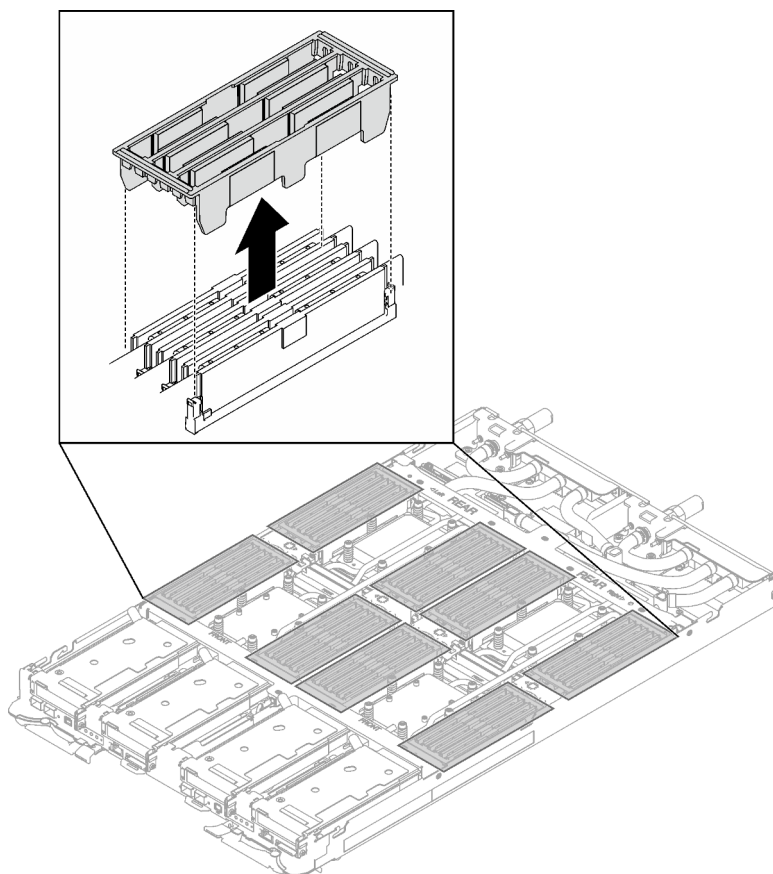
Abbildung 131. Entfernen der DIMM-Abdeckung
