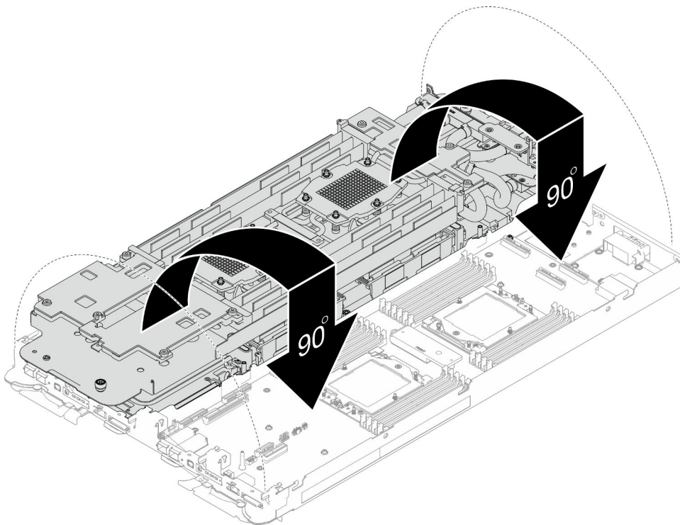
Abbildung 236. Installieren des Wasserkreislaufs
