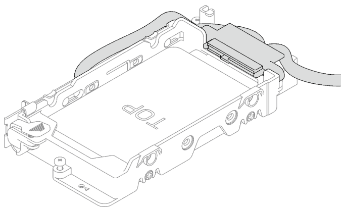
Abbildung 67. Sichern des nicht angeschlossenen Kabelsteckers
