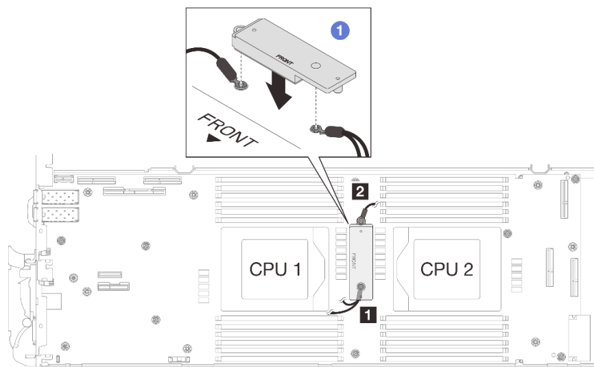
Abbildung 270. Ausrichten der VR-Leiterplatte, geschirmten Kabel und Schraubenlöcher auf der Systemplatine
