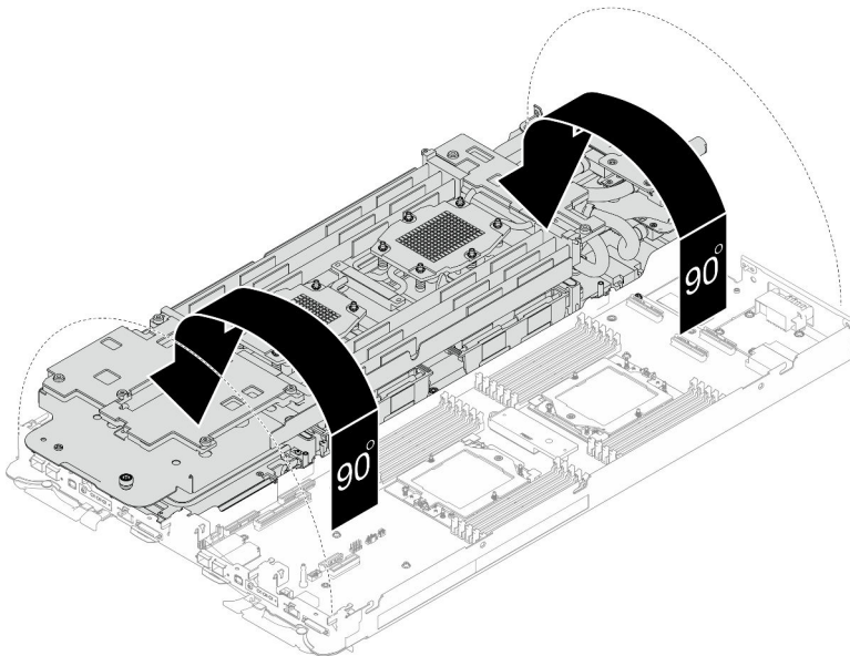
Abbildung 226. Wasserkreislauf falten
