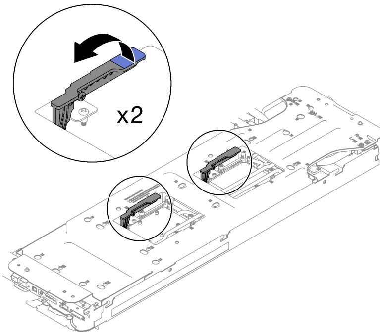
Abbildung 225. Trennen des Wasserkreislaufs vom Prozessor
