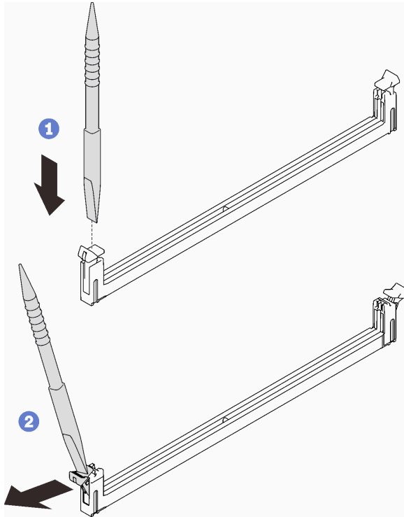
Abbildung 132. Drücken der Halteklammern am Speichermodul-Steckplatz
