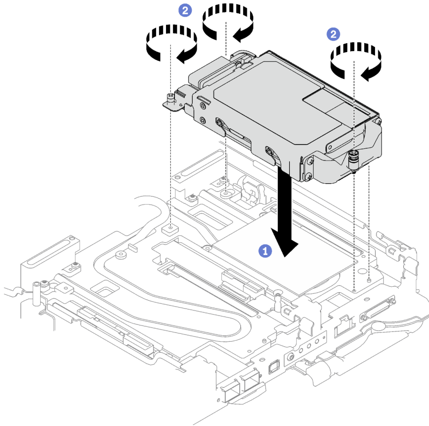
Abbildung 116. Installation einer E3.s-Laufwerkhalterung
