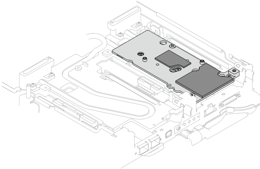
Abbildung 174. Schnittstellen-Pad auf Kühlplatte für CX-7 NDR 200
