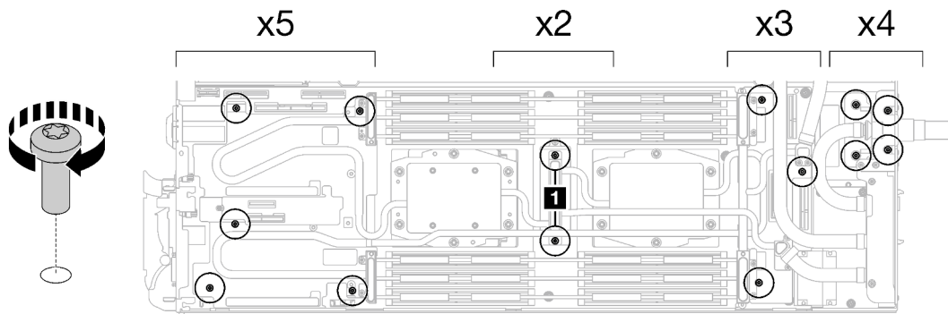
Abbildung 241. Installieren der Schrauben am Wasserkreislauf und Schnellanschluss
