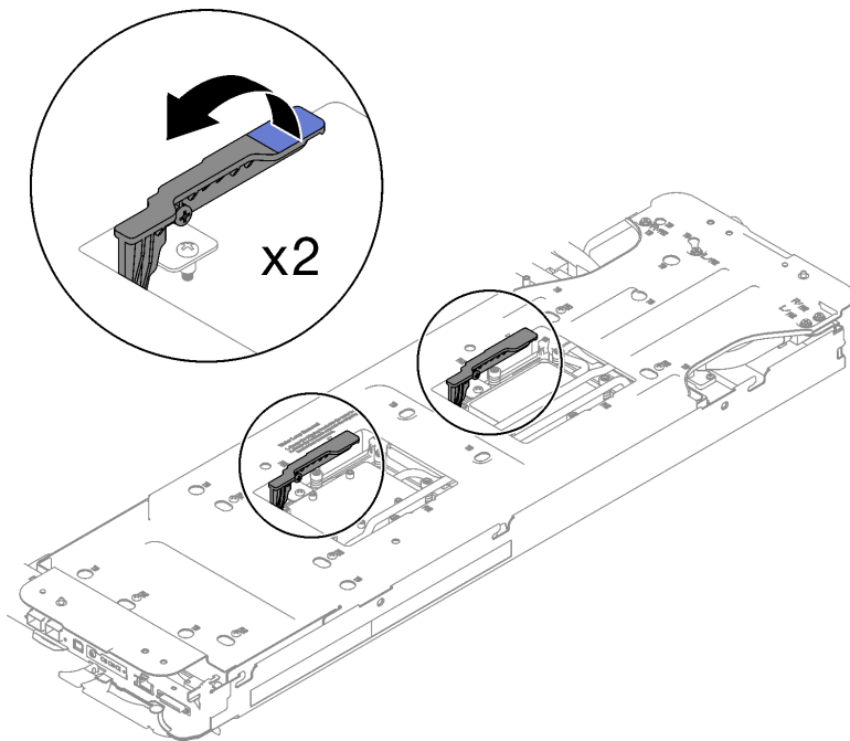
Abbildung 201. Trennen des Wasserkreislaufs vom Prozessor
