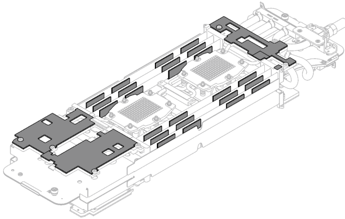
Abbildung 206. Gap-Pads am Wasserkreislauf (Unterseite)
