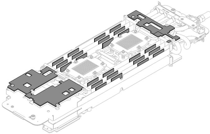
Abbildung 24. Gap-Pads am Wasserkreislauf (Unterseite)
