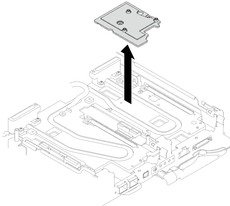
Abbildung 185. Entfernen der Schnittstellenplatte
