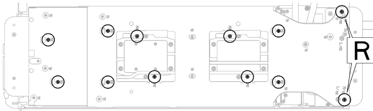
Abbildung 198. Installation der Schrauben der Wasserkreislaufhalterung
