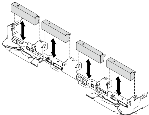
Abbildung 83. Entfernen der Abdeckblende für Frontblende
