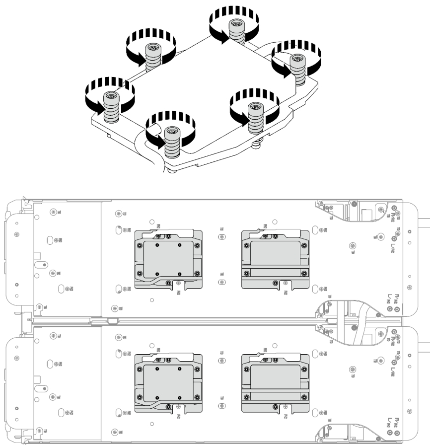
Abbildung 16. Entfernen der Prozessorkühlplatte
