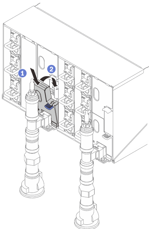
Abbildung 298. Installieren der unteren EMV-Abschirmung
