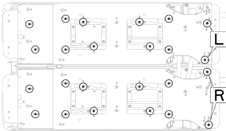
Abbildung 14. Installation der Schrauben der Wasserkreislaufhalterung
