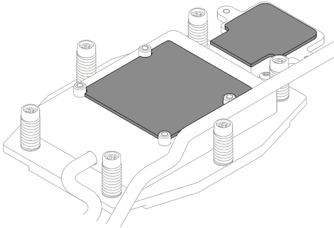
Abbildung 126. Putty-Pads auf der Kühlplatte des Prozessors und der M.2-Rückwandplatine
