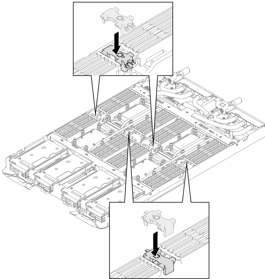
Abbildung 52. Installation des DIMM-Kamms
