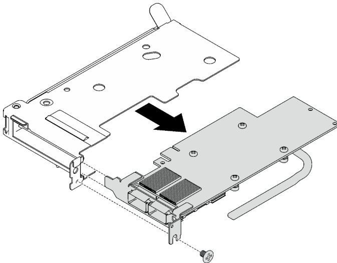
Abbildung 143. Entfernen des PCIe-Adapters
