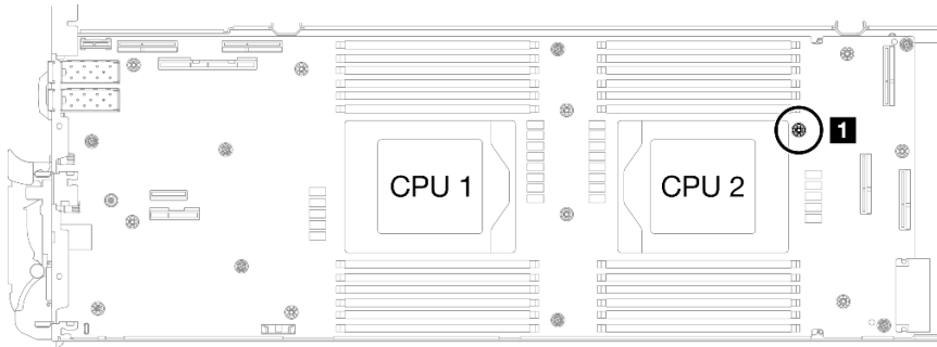
Abbildung 273. Position des Schraubenlochs von geschirmtem Kabel 4
