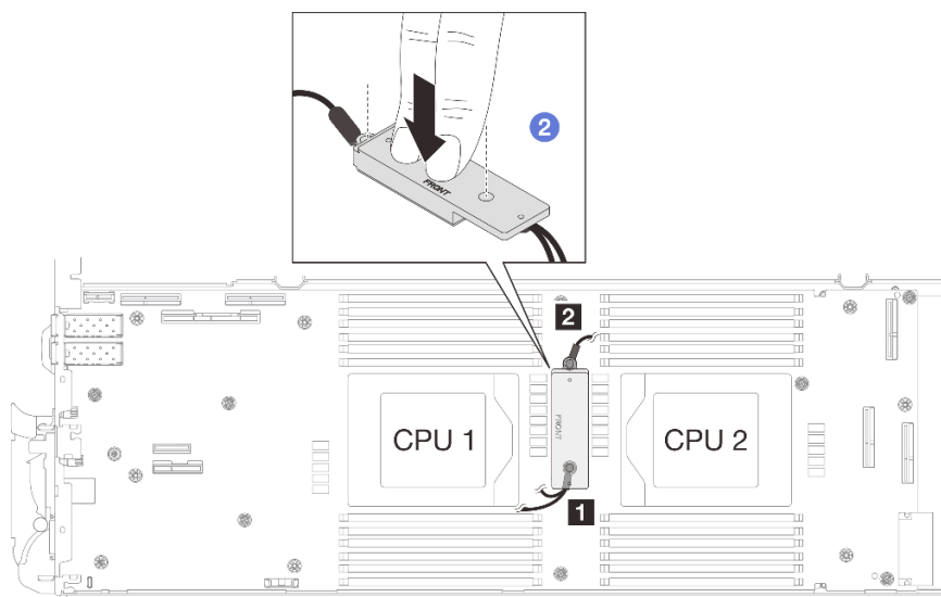
Abbildung 41. Drücken auf die VR-Leiterplatte
