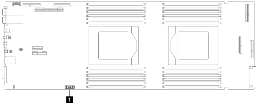
Abbildung 46. Position der CMOS-Batterie
