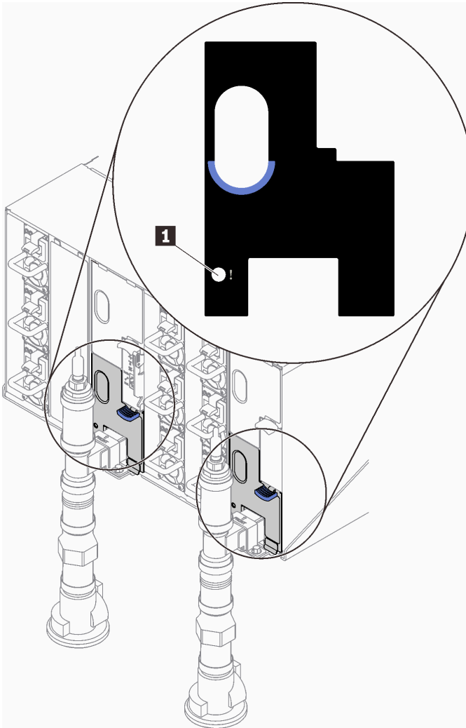
Abbildung 294. Tropfsensor-Anzeige
