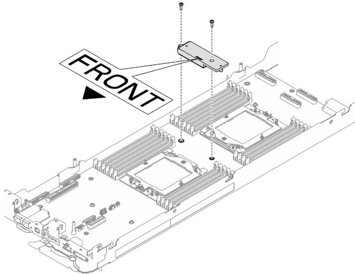
Abbildung 36. Entfernen der VR-Leiterplatte
