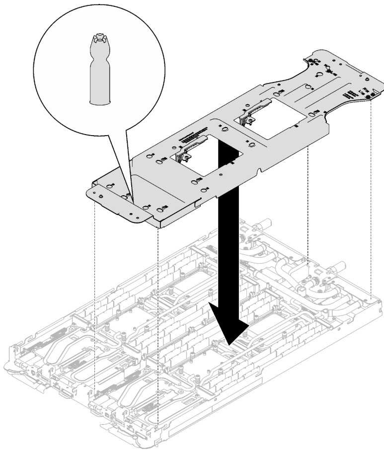
Abbildung 221. Installieren der Wasserkreislaufhalterung
