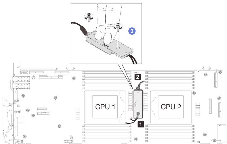
Abbildung 255. Installieren der geschirmten Kabel 1/2 und 3
