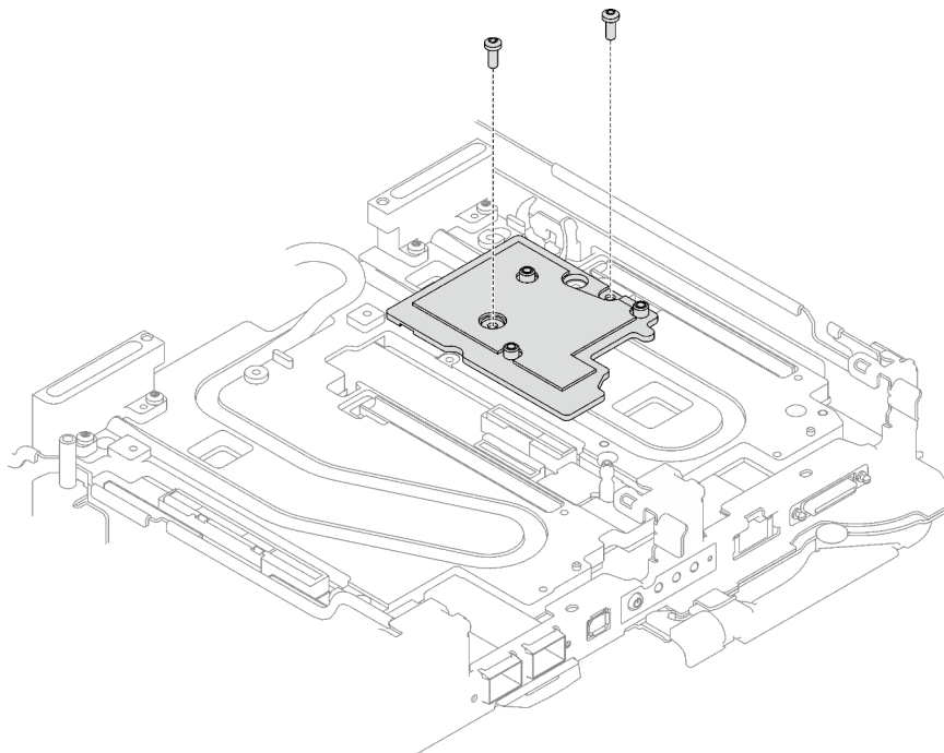
Abbildung 182. Entfernen der Schnittstellenplatte
