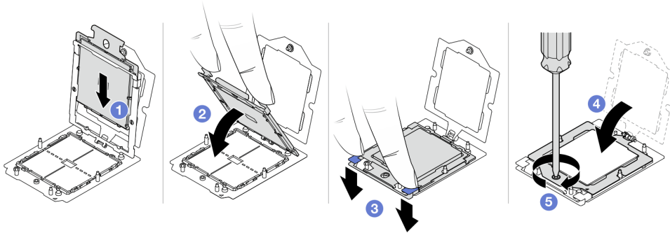
Abbildung 229. Installieren eines Prozessors
