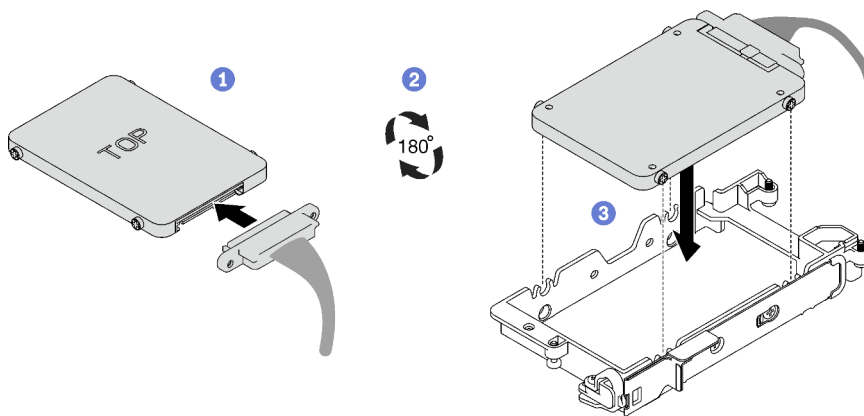
Abbildung 65. Installation des 7-mm-Laufwerks
