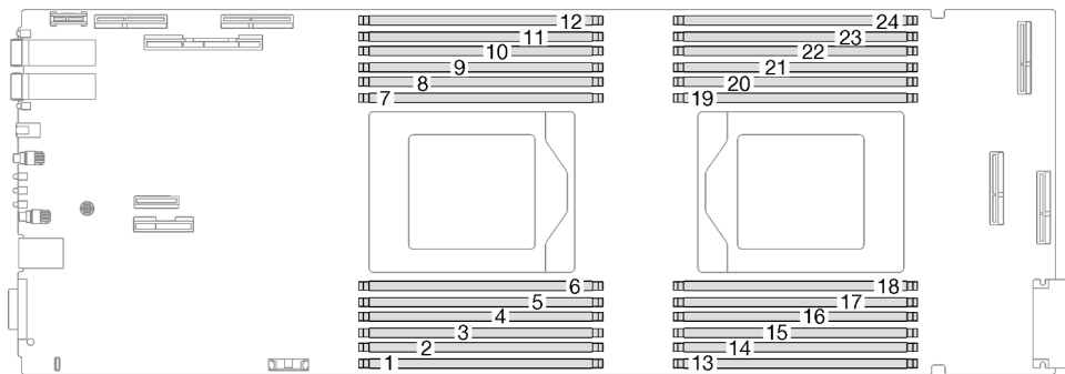
Abbildung 129. Position der Speichermodul-Anschlüsse
