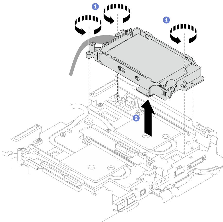
Abbildung 58. Entfernen der Laufwerkhalterung mit einem 15-mm-Laufwerk
