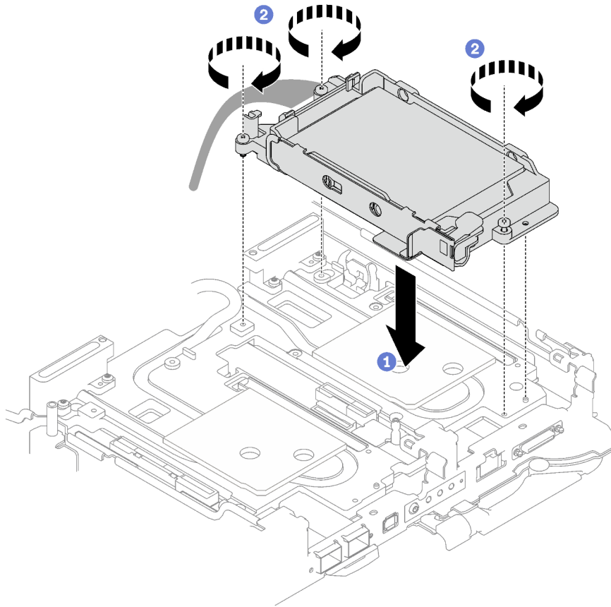
Abbildung 78. Installation einer Laufwerkhalterung mit 15-mm-Laufwerk
