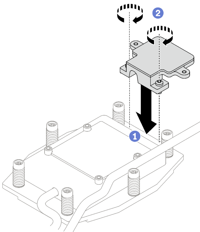
Abbildung 125. Installieren der Kühlplatte der M.2-Rückwandplatine
