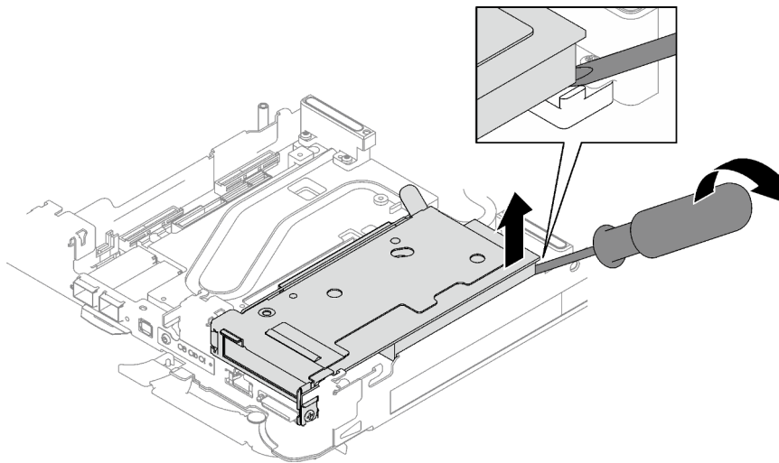
Abbildung 180. Lösen des PCIe-Adapterrahmens von der Kühlplatte des Wasserkreislaufs
