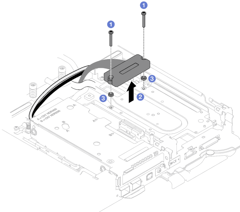
Abbildung 162. Entfernen des Verbindungskabels
