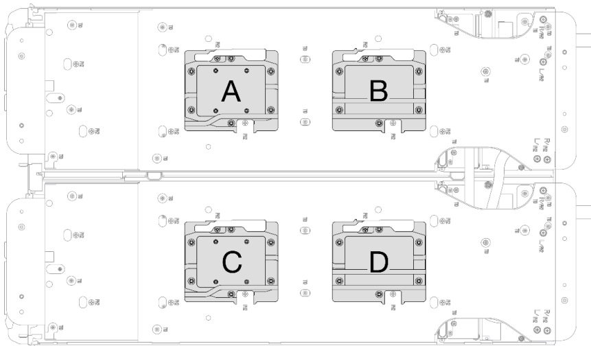
Abbildung 30. Installieren der Prozessorkühlplatte
