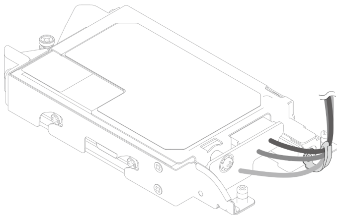
Abbildung 112. Bündeln von Kabeln mit Kabelbinder
