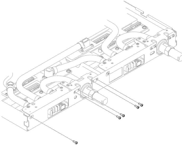
Abbildung 216. Installation der Schrauben am Schnellanschluss
