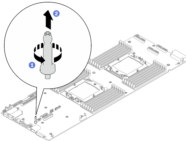
Abbildung 247. Entfernen des Führungsstifts
