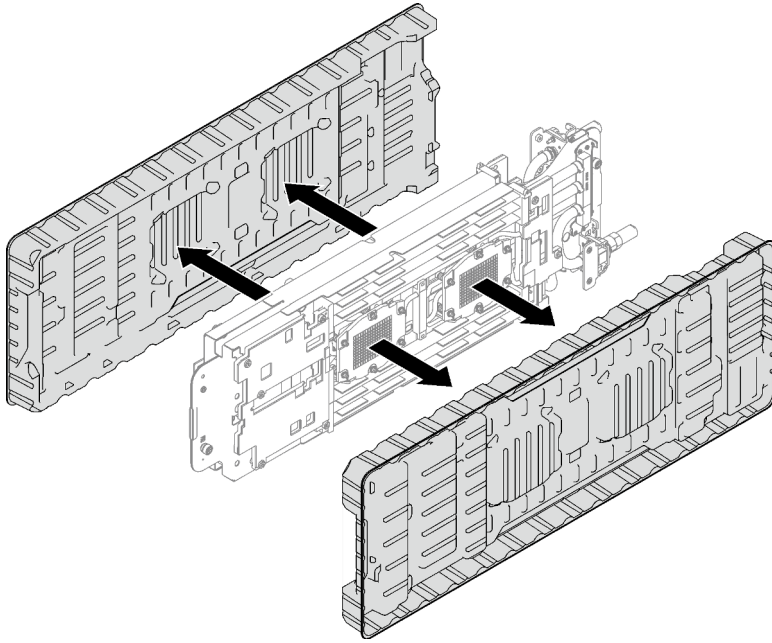
Abbildung 22. Entfernen der Kunststoffabdeckungen der Wärmeleitpaste
