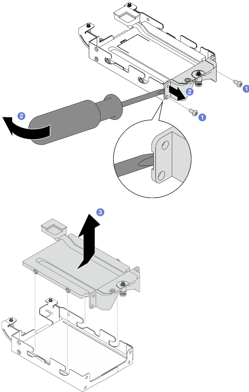
Abbildung 103. Entfernen der Leitplatte
