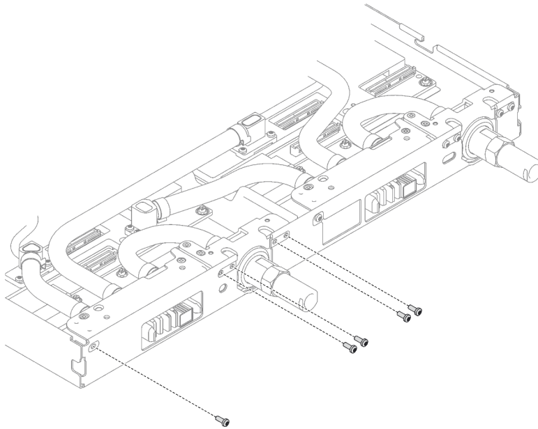
Abbildung 242. Installation der Schrauben am Schnellanschluss
