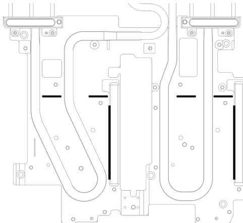
Abbildung 114. Markierungen auf dem Wasserkreislauf für die Ausrichtung des E3.S-Gap-Pad
