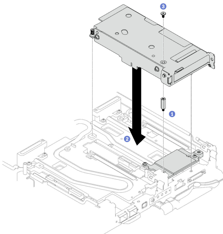
Abbildung 159. PCIe-Adapterkartenbaugruppe installieren
