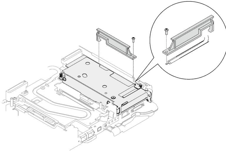
Abbildung 149. Entfernen des Wärmerohrträgers
