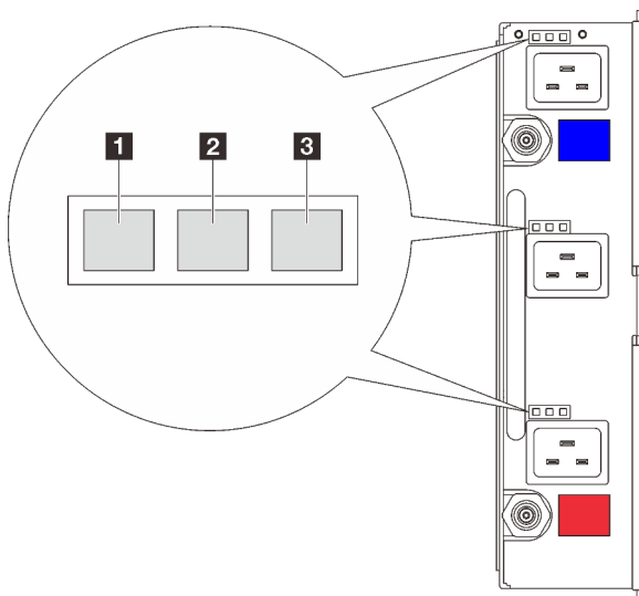
Abbildung 291. DWC Netzteilanzeigen
