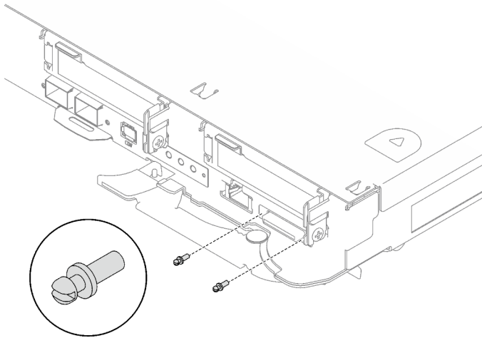
Abbildung 243. Entfernen der KVM-Schrauben
