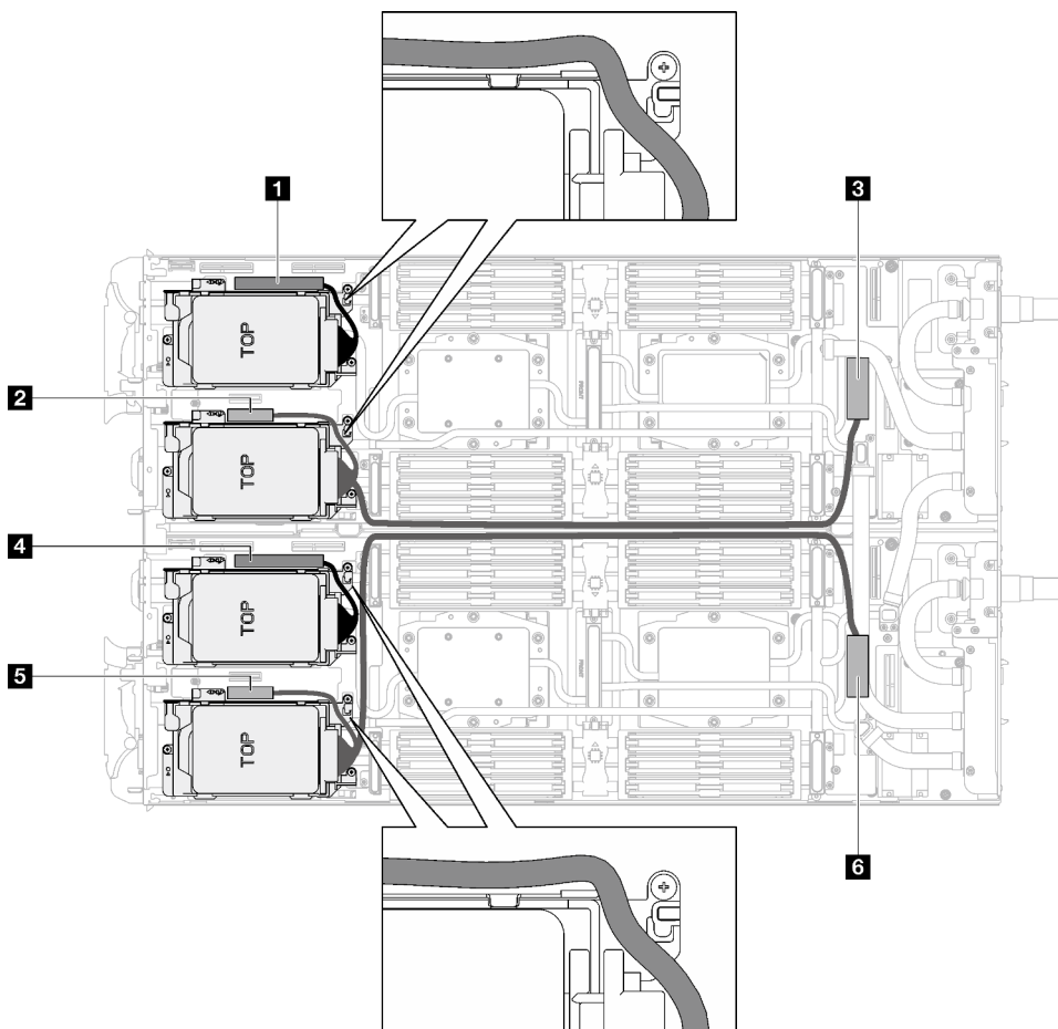
Abbildung 54. Kabelführung der Laufwerkbaugruppe für SATA-Laufwerke
