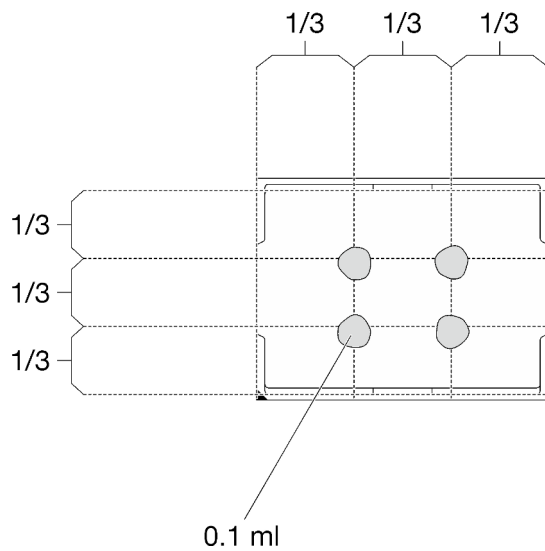
Abbildung 230. Auftragen der Wärmeleitpaste
