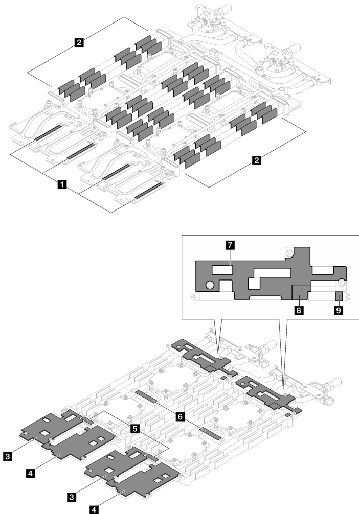
Abbildung 2. Wasserkreislauf – Identifikation und Position der Gap-Pads und Putty-Pads
