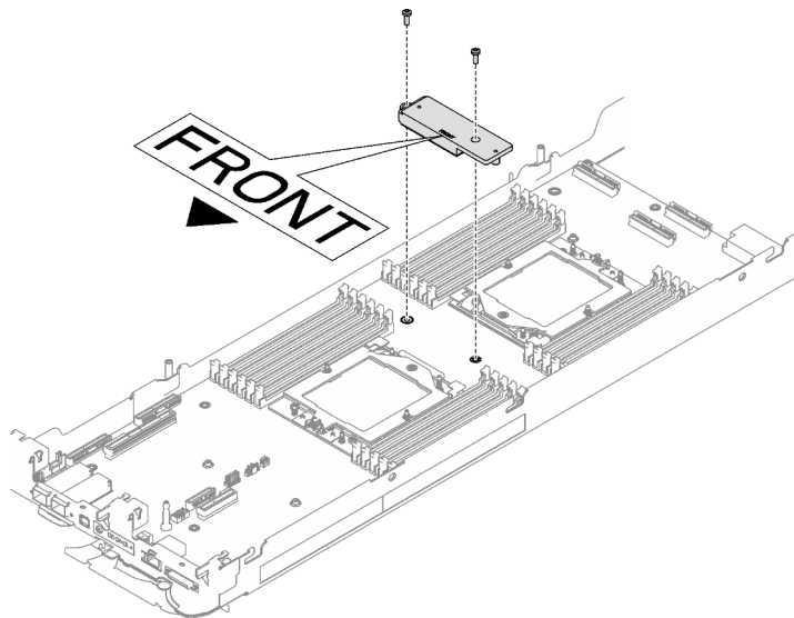
Abbildung 43. Entfernen der VR-Leitplatte
