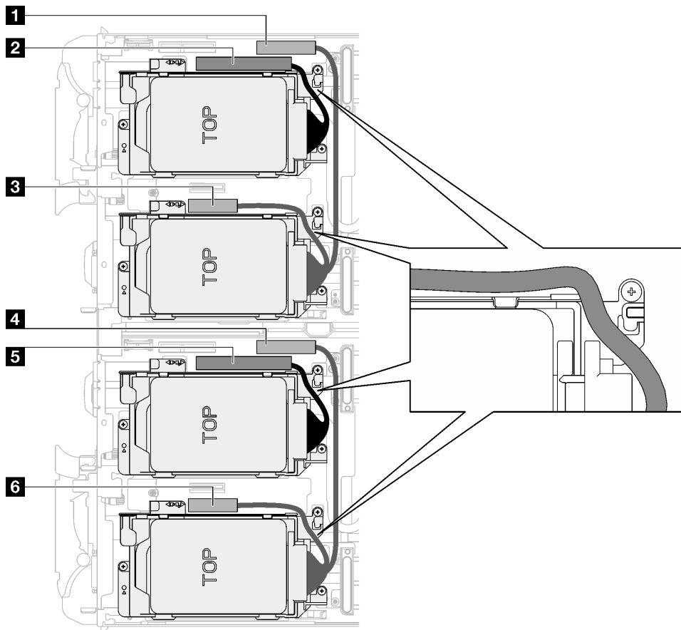
Abbildung 81. Kabelführung der Laufwerkbaugruppe für alle NVMe-Laufwerke
