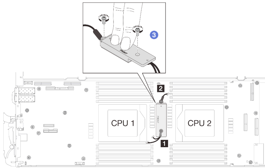
Abbildung 42. Installieren der geschirmten Kabel 1/2 und 3
