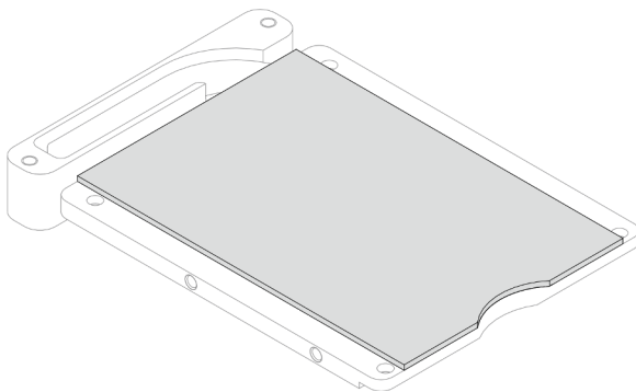
Abbildung 86. Installation des Gap-Pads auf der Leitplatte
