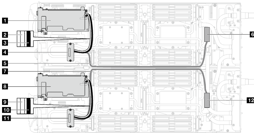
Abbildung 284. Kabelführung für die Socket Direct-Konfiguration
