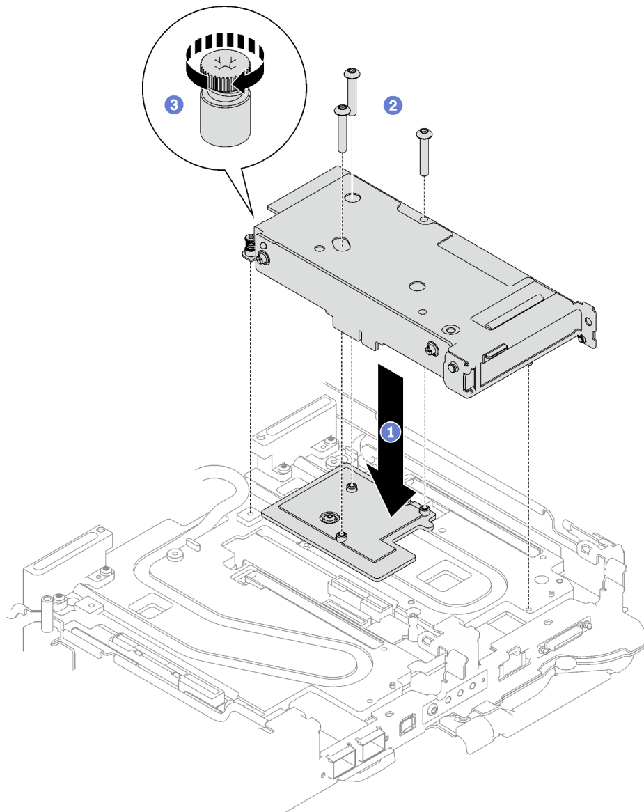
Abbildung 192. PCIe-Adapterkartenbaugruppe installieren
