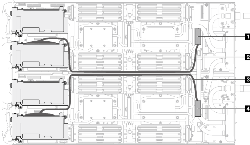
Abbildung 282. Ausgewogene E/A-Konfiguration
