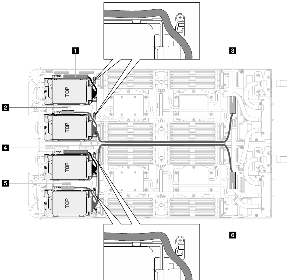
Abbildung 79. Kabelführung der Laufwerkbaugruppe für SATA-Laufwerke
