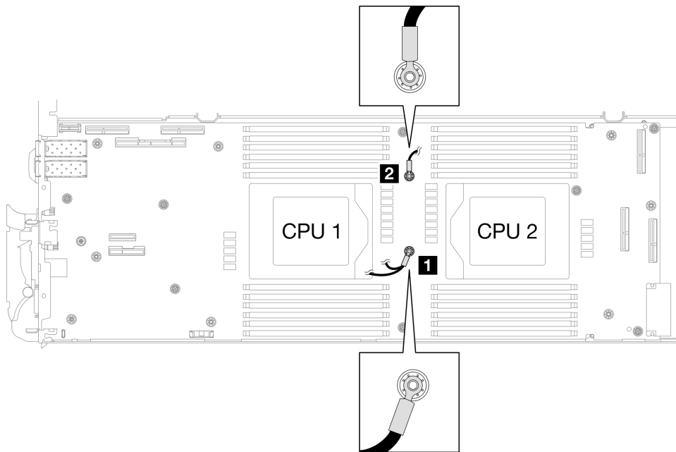
Abbildung 39. Ausrichten von abgeschirmtem Kabel 1/2 und abgeschirmtem Kabel 3 mit Schraubenlöchern
