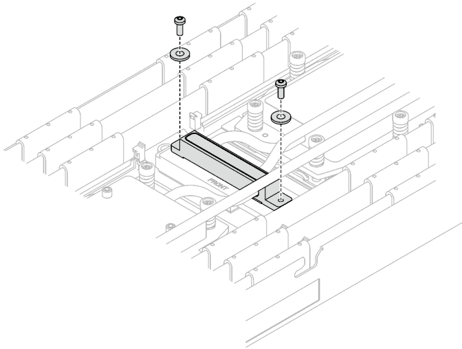
Abbildung 33. Schrauben der VR-Kühlplatte mit Unterlegscheiben
