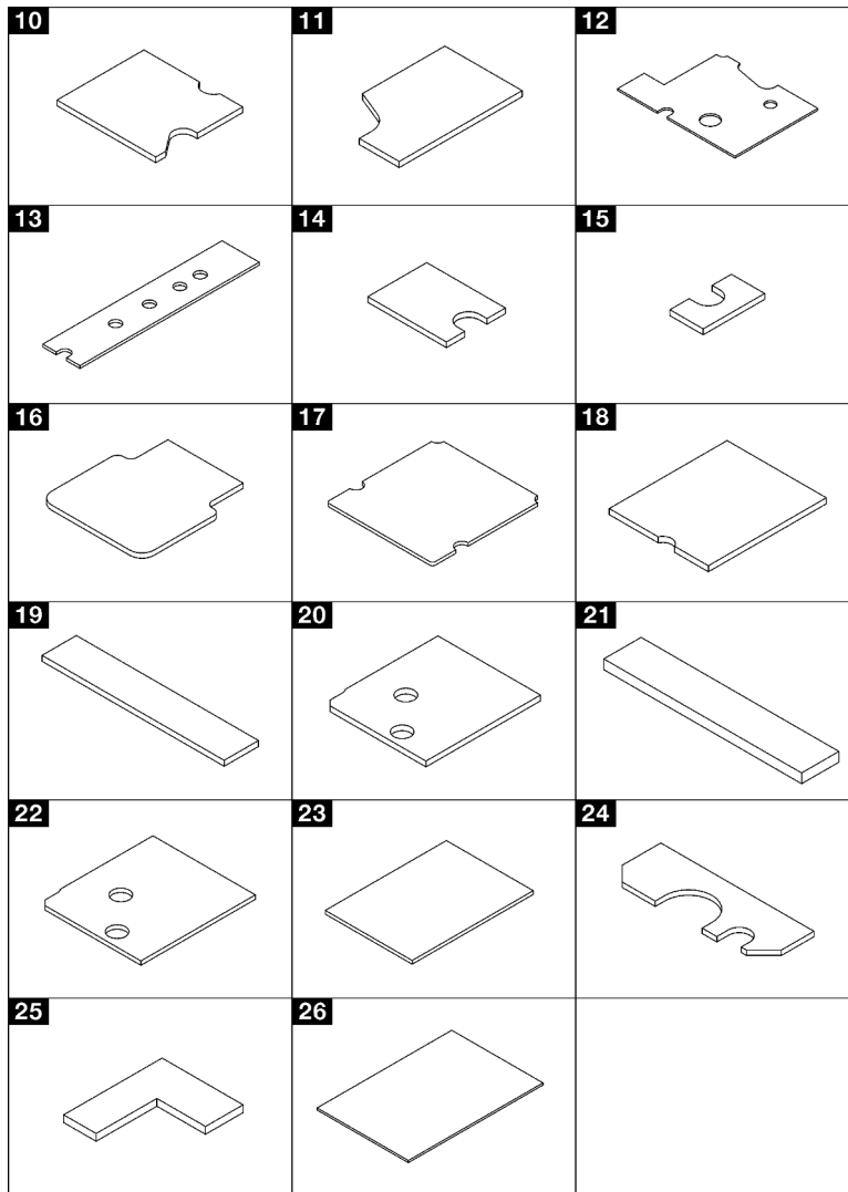
Abbildung 3. Komponenten – Identifikation und Position von Gap-Pad/Putty-Pad
