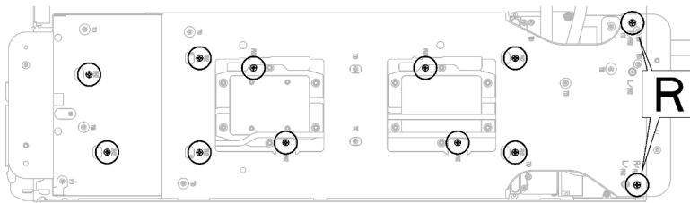
Abbildung 212. Lösen der Schrauben der Wasserkreislaufhalterung
