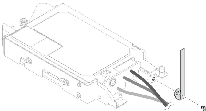
Abbildung 111. Kabelbinder-Installation
