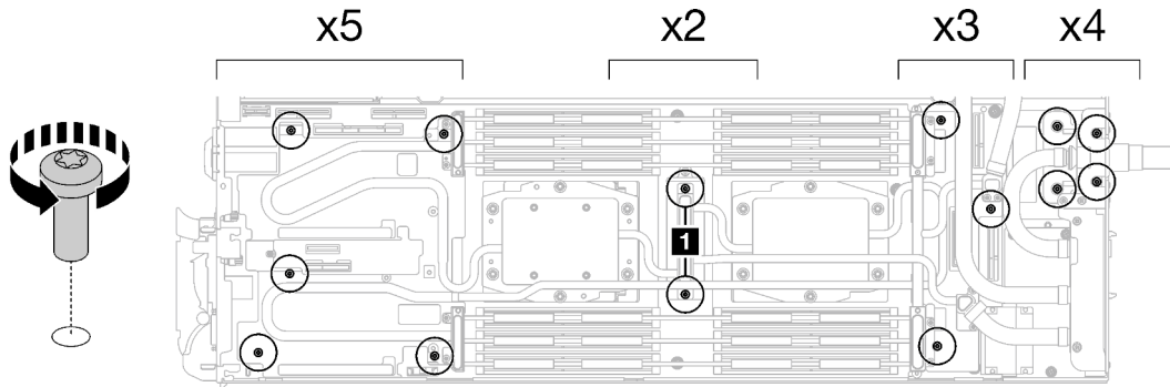
Abbildung 12. Entfernen der Schrauben des Wasserkreislaufs
