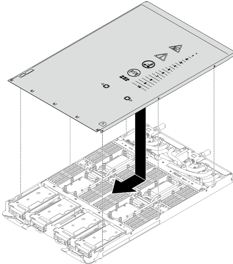
Abbildung 7. Installation der Abdeckung für Einbaurahmen
