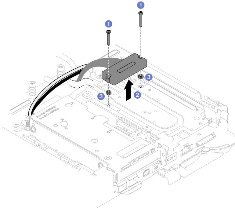
Abbildung 178. Entfernen des Verbindungskabels
