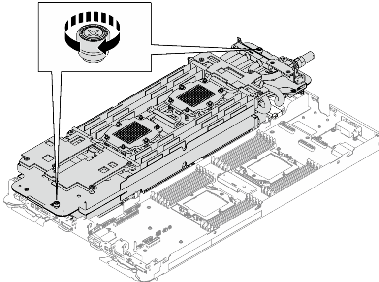
Abbildung 19. Anziehen der Rändelschrauben
