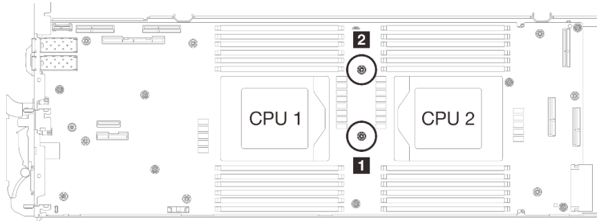
Abbildung 38. Position der Schraubenlöcher von geschirmtem Kabel 1/2 und 3
