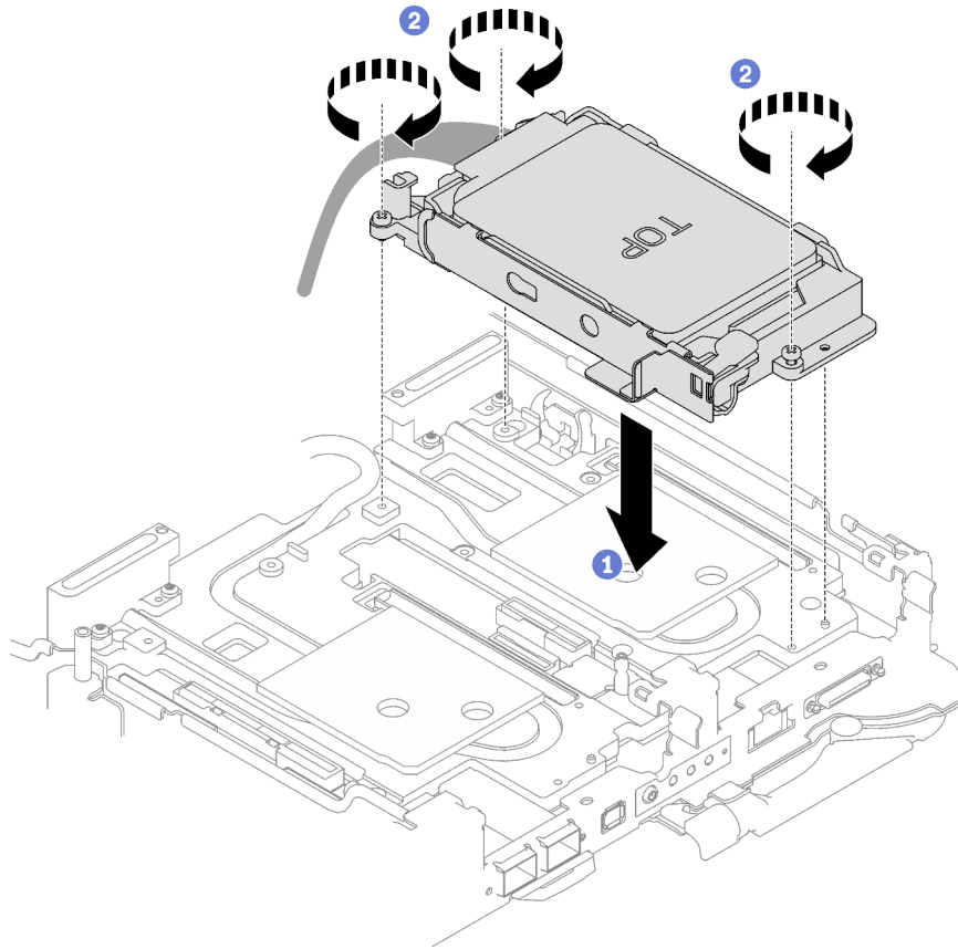
Abbildung 77. Installation einer Laufwerkhalterung mit zwei 7-mm-Laufwerken
