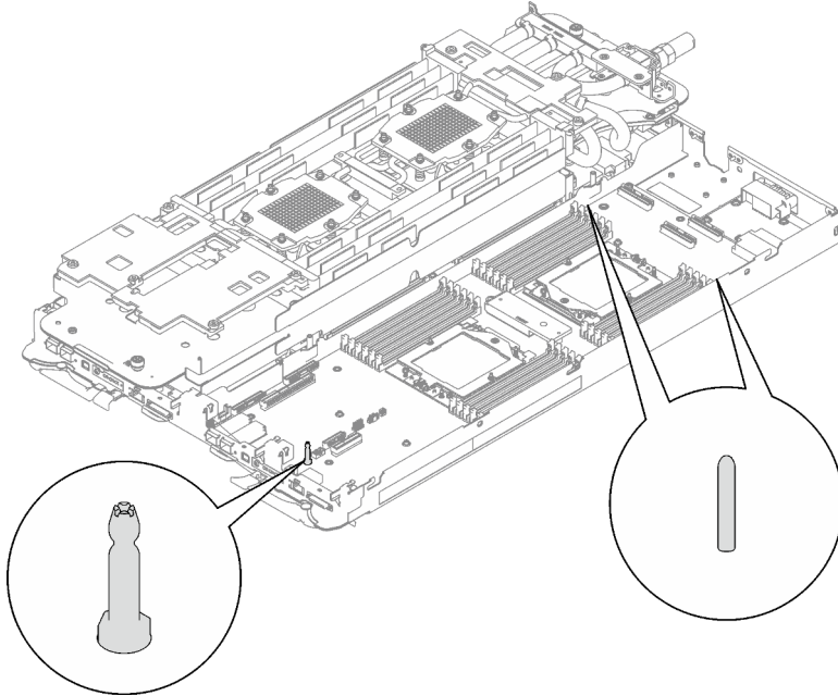
Abbildung 235. Führungsstifte an der rechten Seite des Rechenknotens
