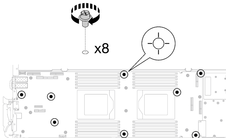
Abbildung 280. Anbringen der Systemplatinschrauben
