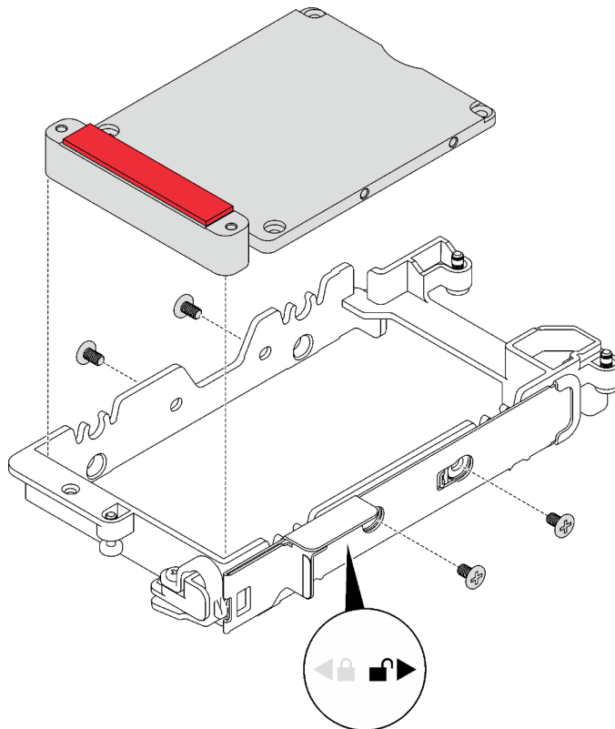
Abbildung 64. Entfernen der Leitplatte
