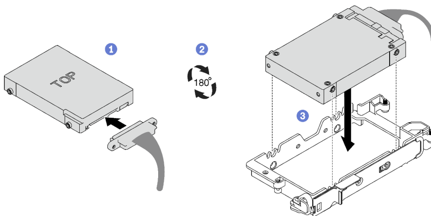
Abbildung 66. Installation des 15-mm-Laufwerks
