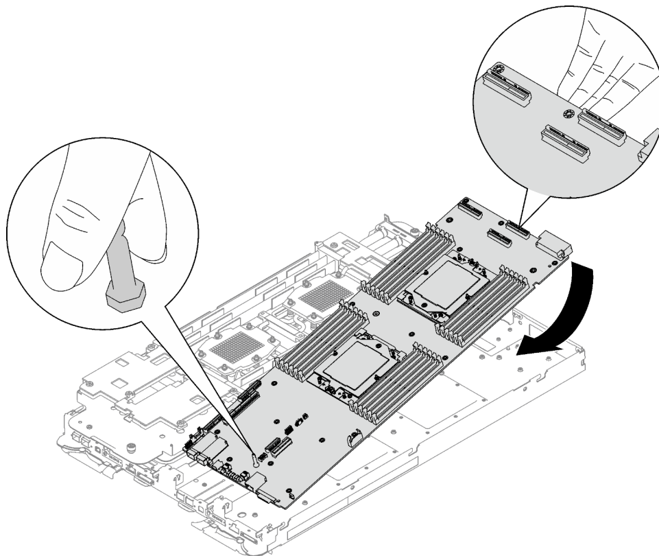
Abbildung 249. Systemplatineeinbau
