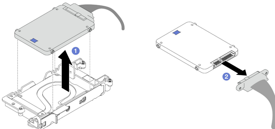
Abbildung 85. Entfernen des unteren Laufwerks
