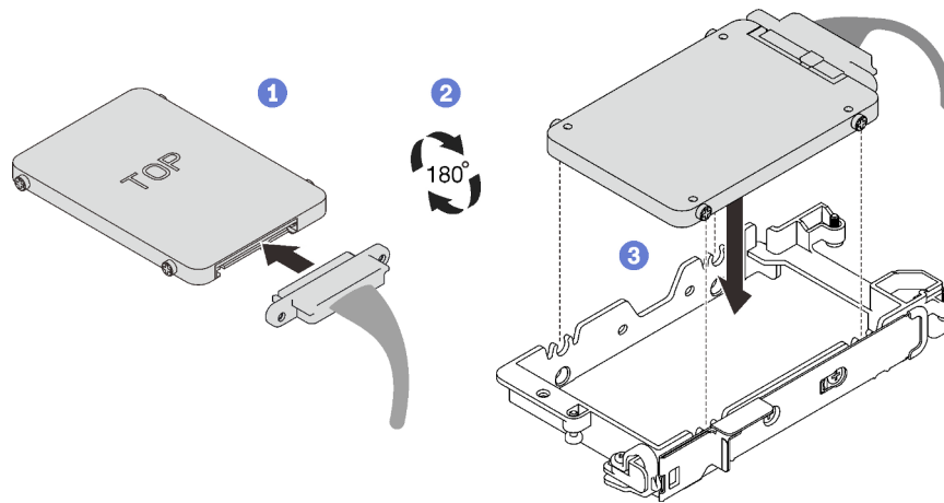
Abbildung 69. Installation des unteren Laufwerks
