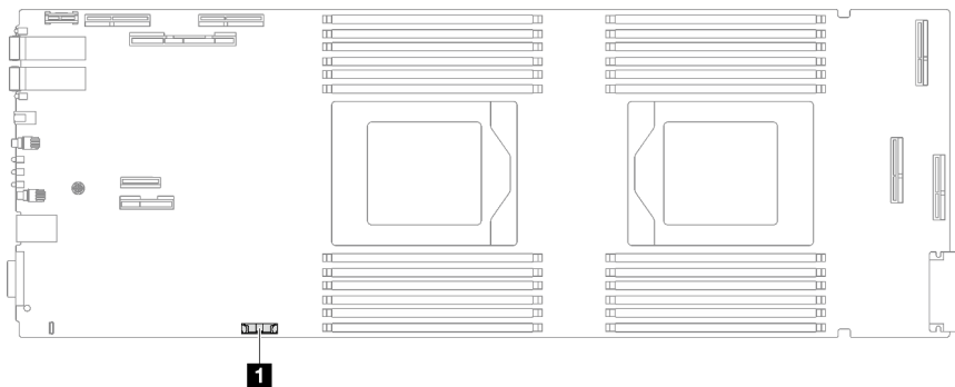
Abbildung 48. Position der CMOS-Batterie
