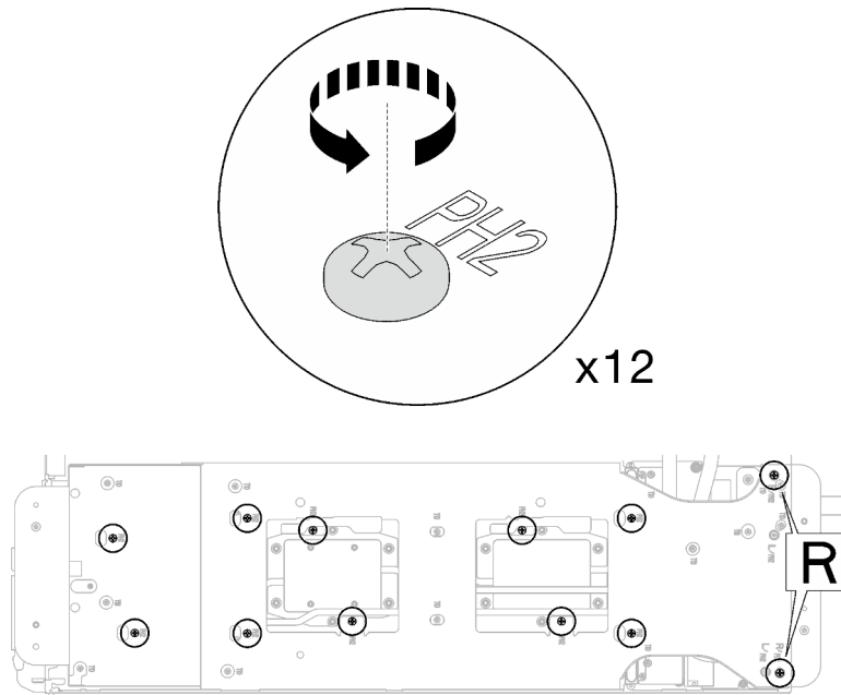
Abbildung 238. Lösen der Schrauben der Wasserkreislaufhalterung
