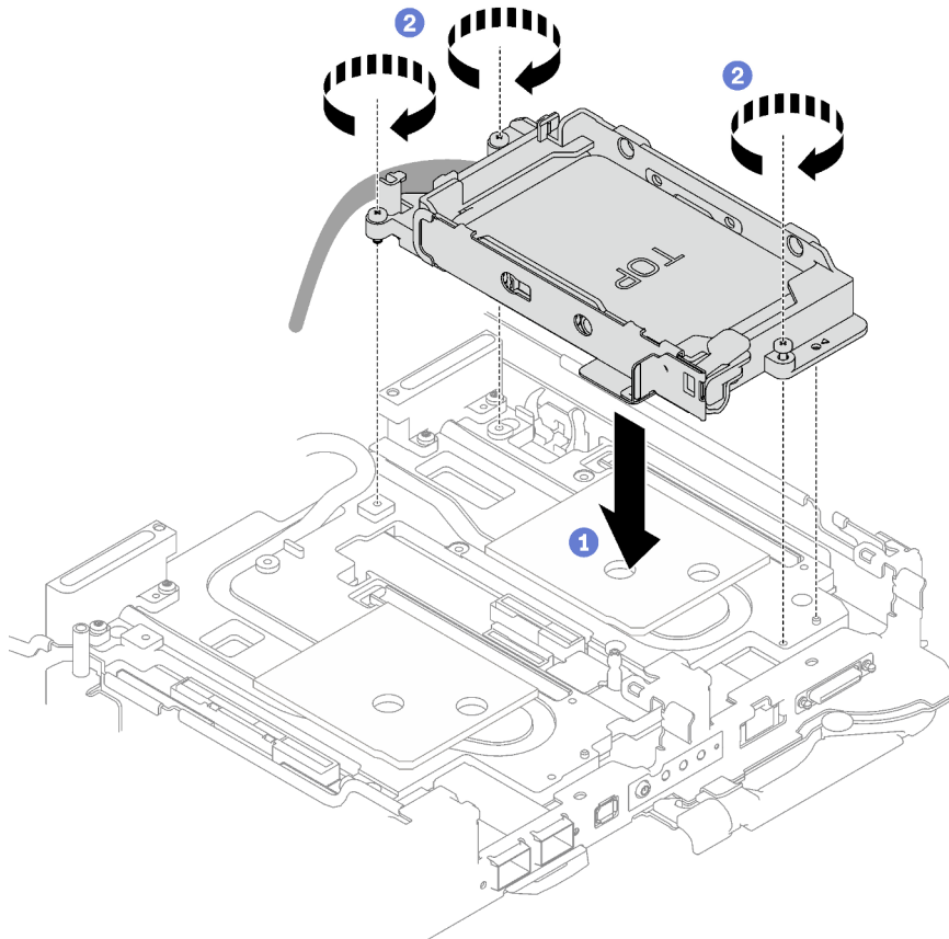
Abbildung 76. Installation einer Laufwerkhalterung mit 7-mm-Laufwerk
