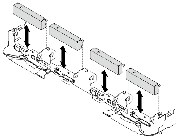
Abbildung 59. Entfernen der Abdeckblende für Frontblende
