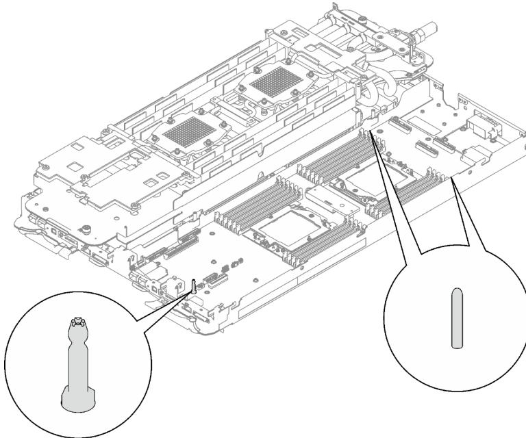
Abbildung 209. Führungstifte an der rechten Seite des Rechenknotens
