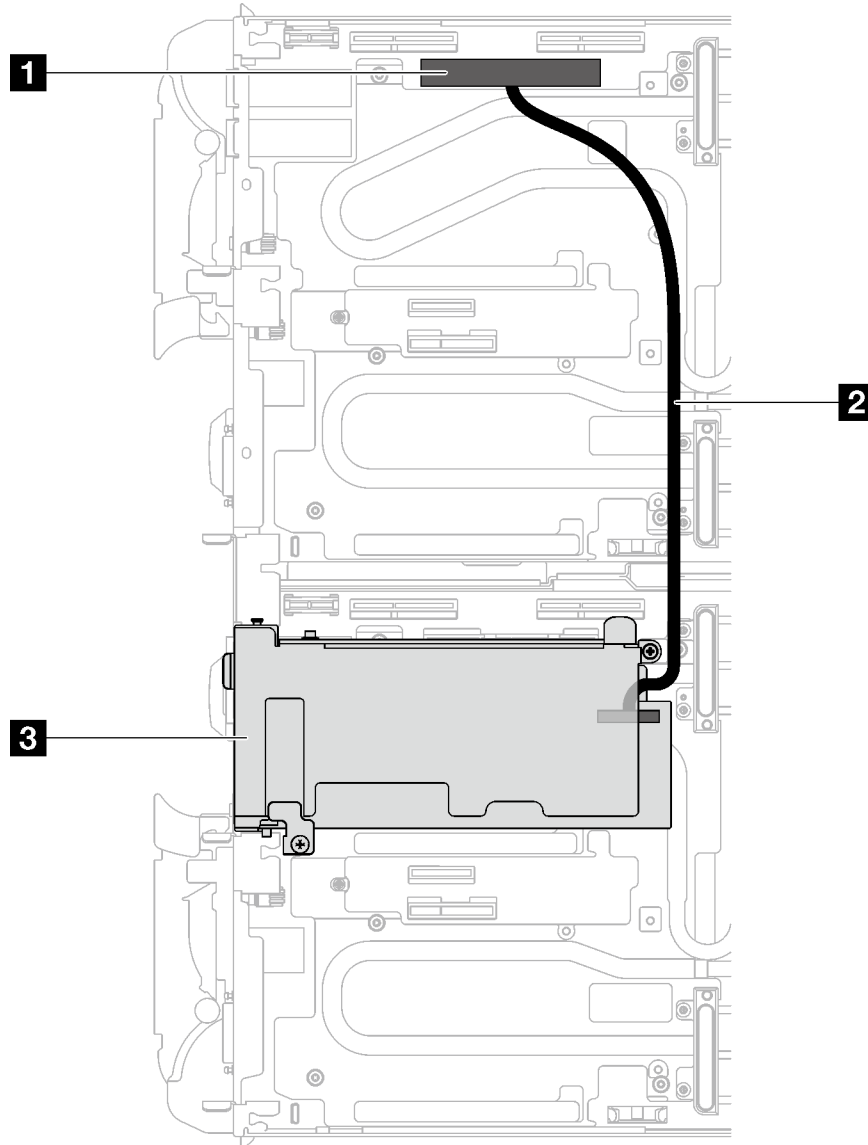
Abbildung 283. Gemeinsam genutzte E/A-Konfiguration
