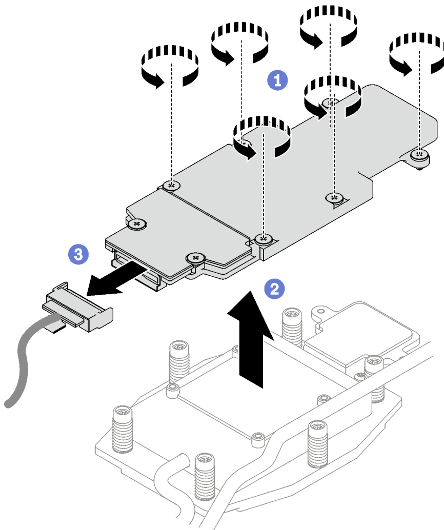
Abbildung 119. Entfernen der M.2-Rückwandplattenbaugruppe
