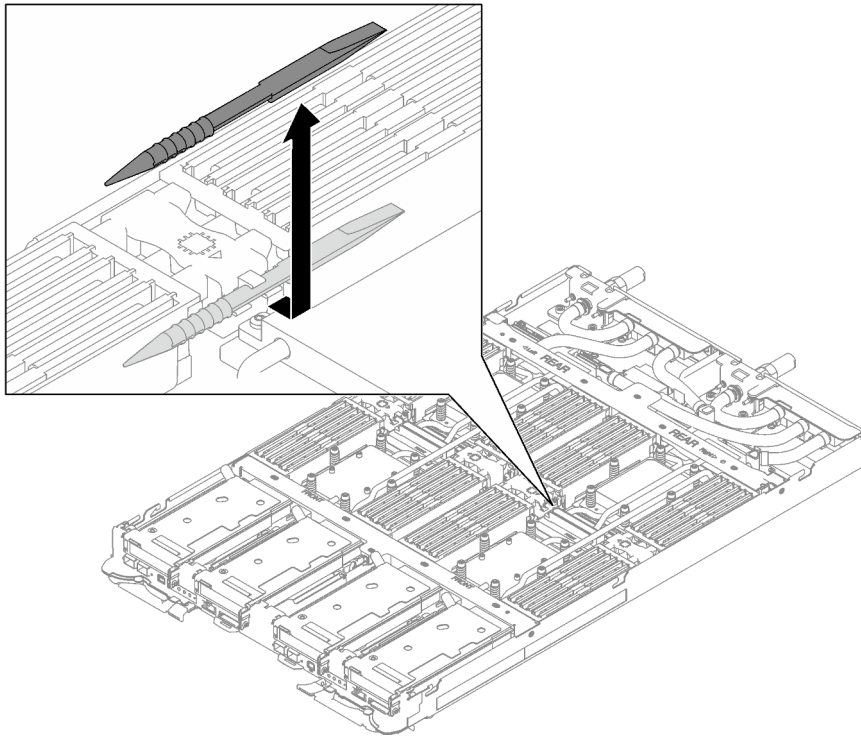
Abbildung 130. Entfernen des Speichermodul-Werkzeugs
