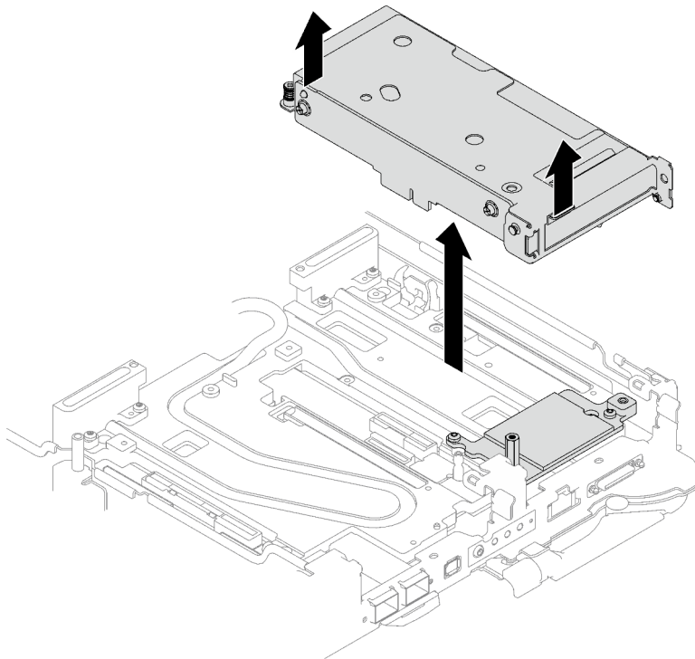
Abbildung 151. Lösen der PCIe-Adapterbaugruppe
