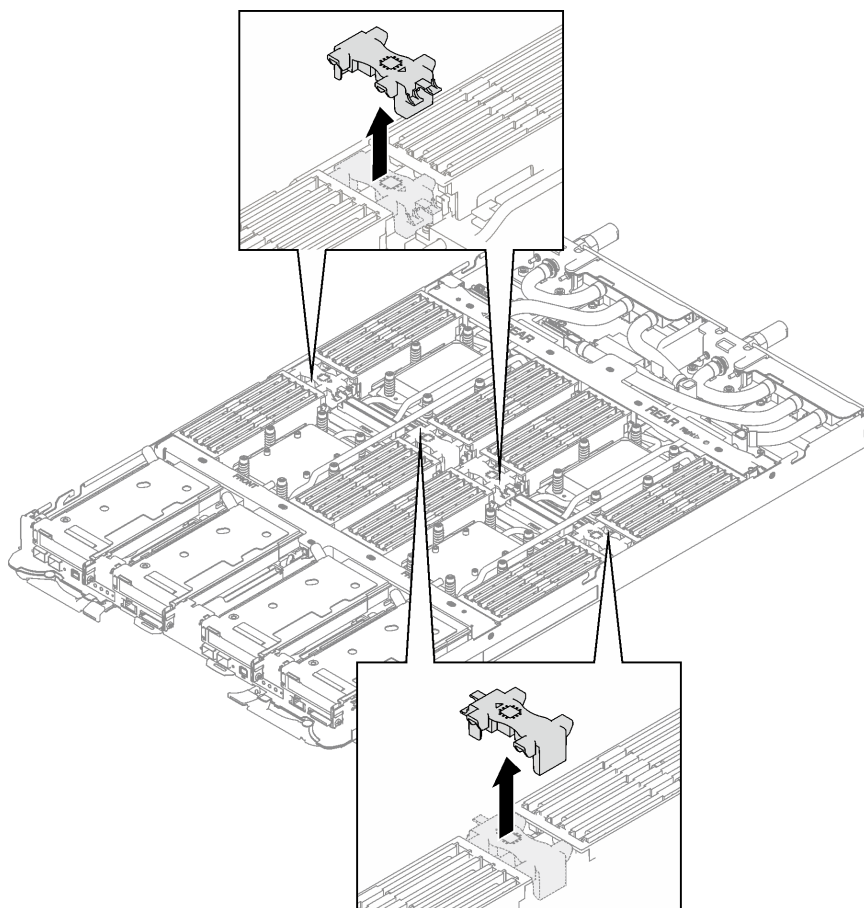
Abbildung 51. Entfernen des DIMM-Kamms
