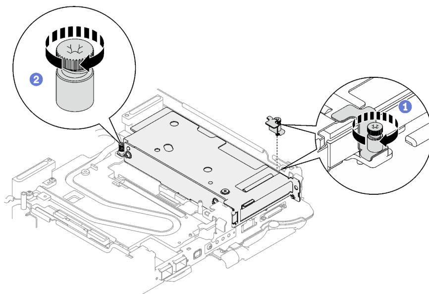
Abbildung 160. Installation der unverlierbaren Schraube der Klemmbefestigung
