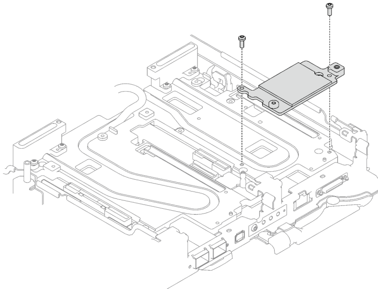
Abbildung 157. Installation der Schnittstellenplatte
