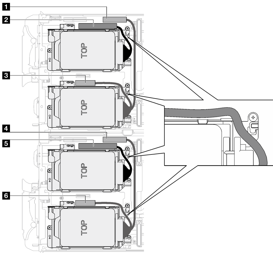
Abbildung 80. Kabelführung der Laufwerkbaugruppe für alle NVMe-Laufwerke
