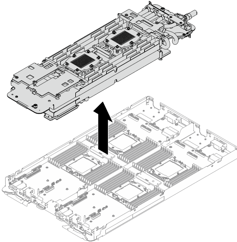
Abbildung 20. Entfernen des Wasserkreislaufs
