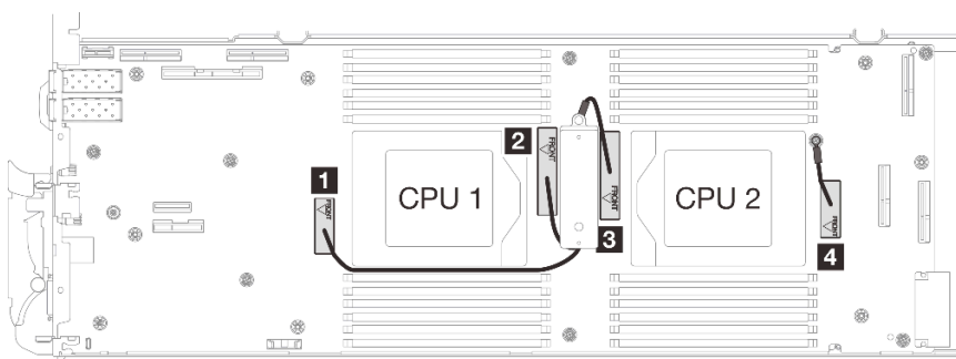
Abbildung 265. Kabelführung für Abschirmrahmen
