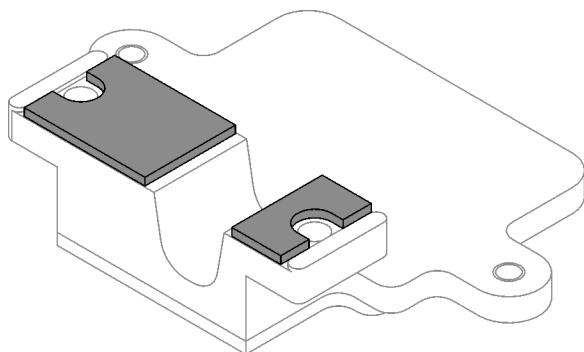
Abbildung 124. Putty-Pads auf der M.2-Rückwandplatine (Unterseite)
