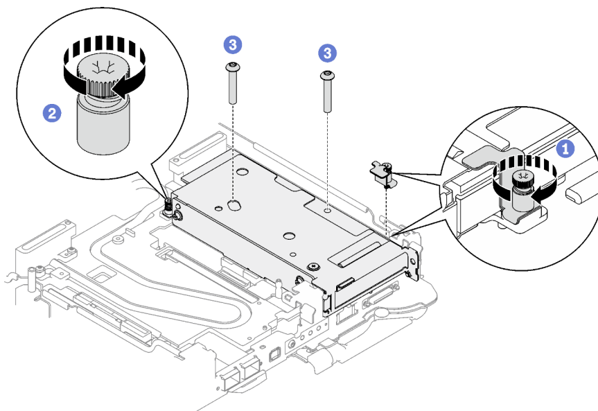
Abbildung 176. Installation der unverlierbaren Schraube der Klemmbefestigung
