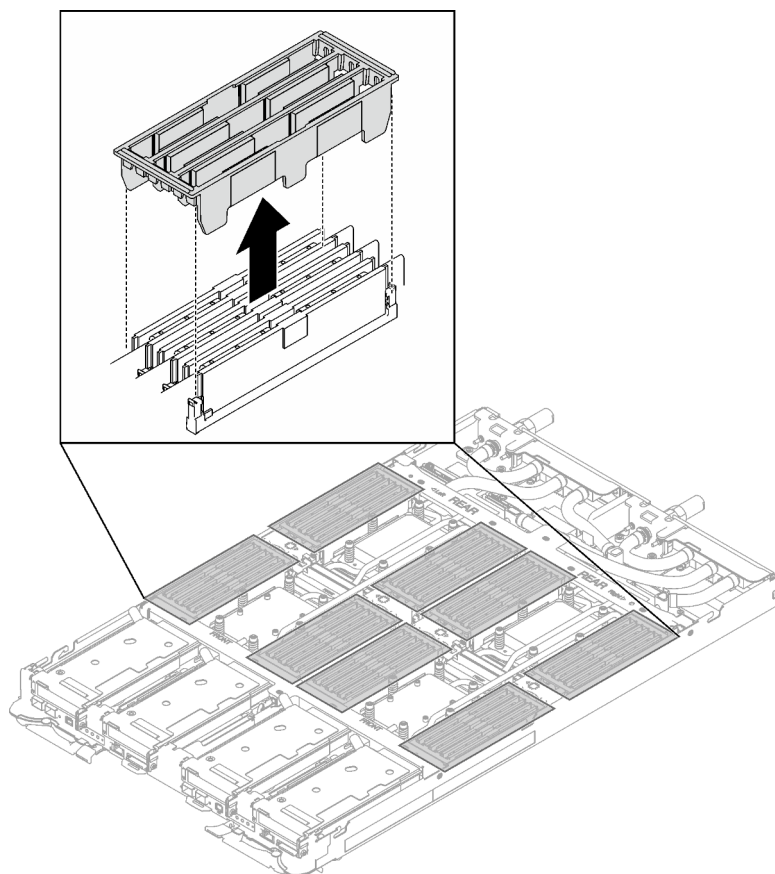
Abbildung 138. Entfernen der DIMM-Abdeckung
