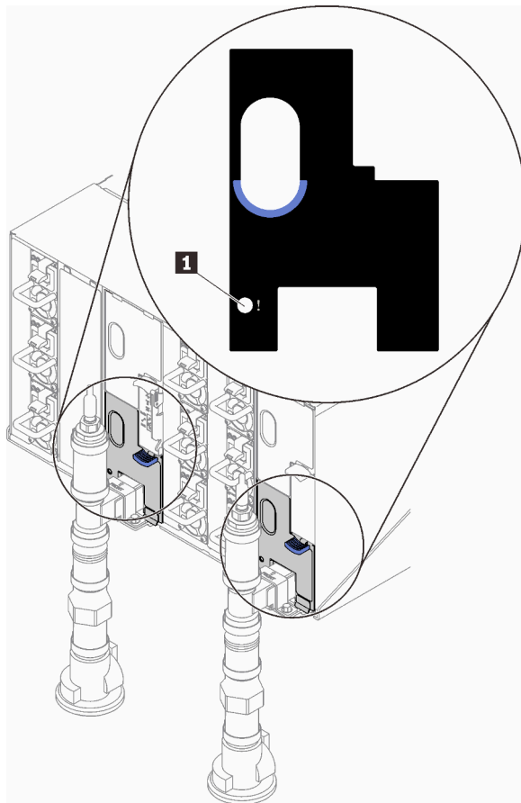
Abbildung 292. Tropfsensor-Anzeige
