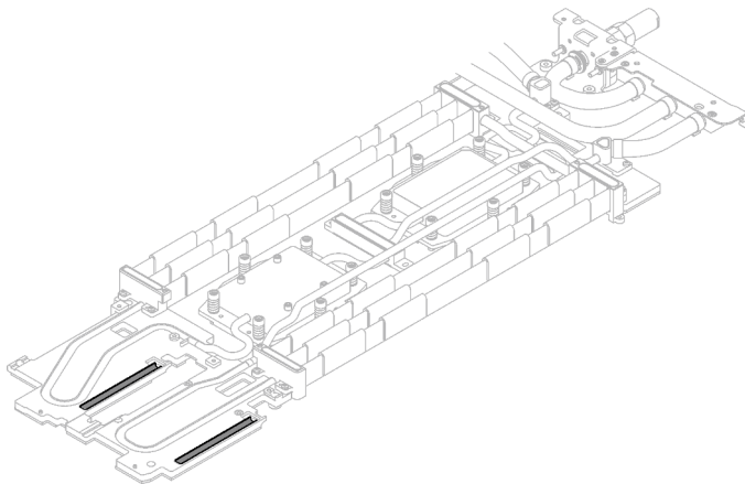
Abbildung 25. Gap-Pads am Wasserkreislauf (Oberseite)
