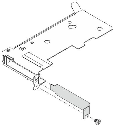
Abbildung 146. Entfernen der Abdeckblende
