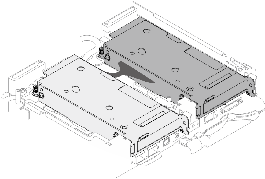
Abbildung 171. Typen von PCIe-Adapterkarten, die in Steckplatz 1 und Steckplatz 2 installiert sind
