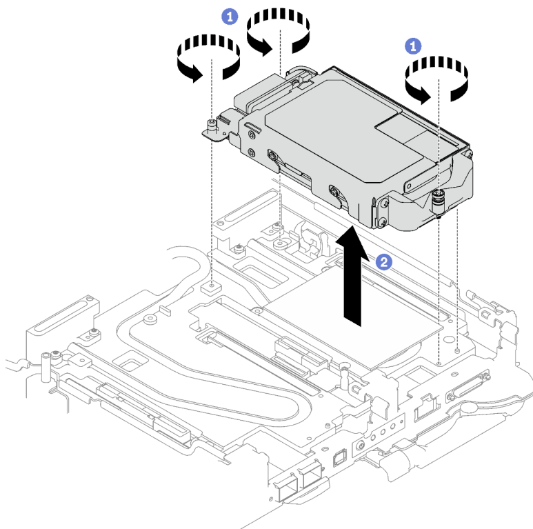
Abbildung 97. E3.s-Laufwerkhalterungsbaugruppe entfernen
