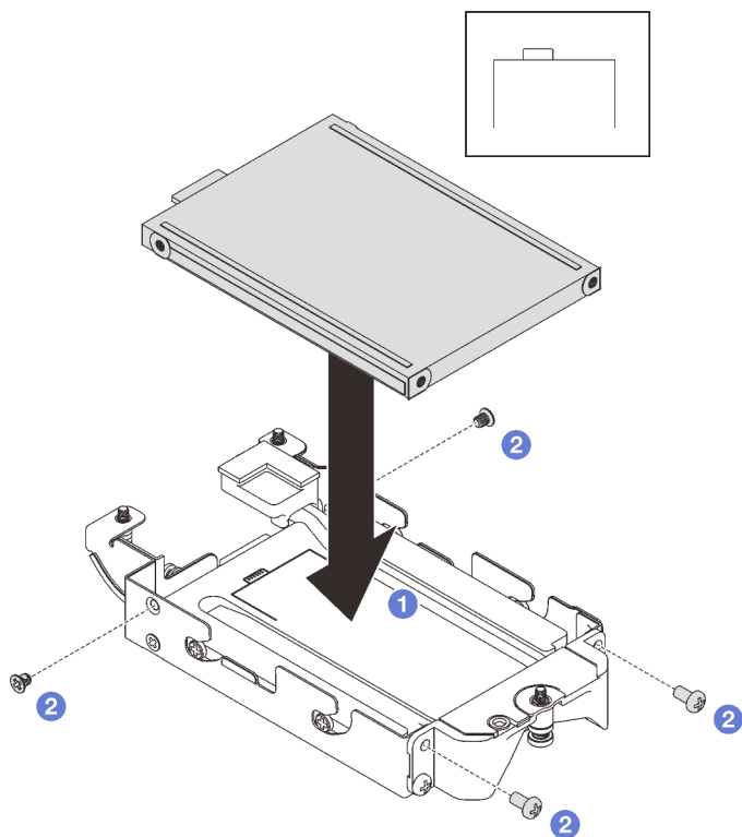
Abbildung 109. Installation des unteren E3.S-Laufwerks
