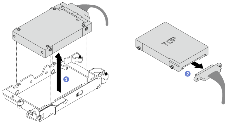
Abbildung 61. Entfernen eines 15-mm-Laufwerks
