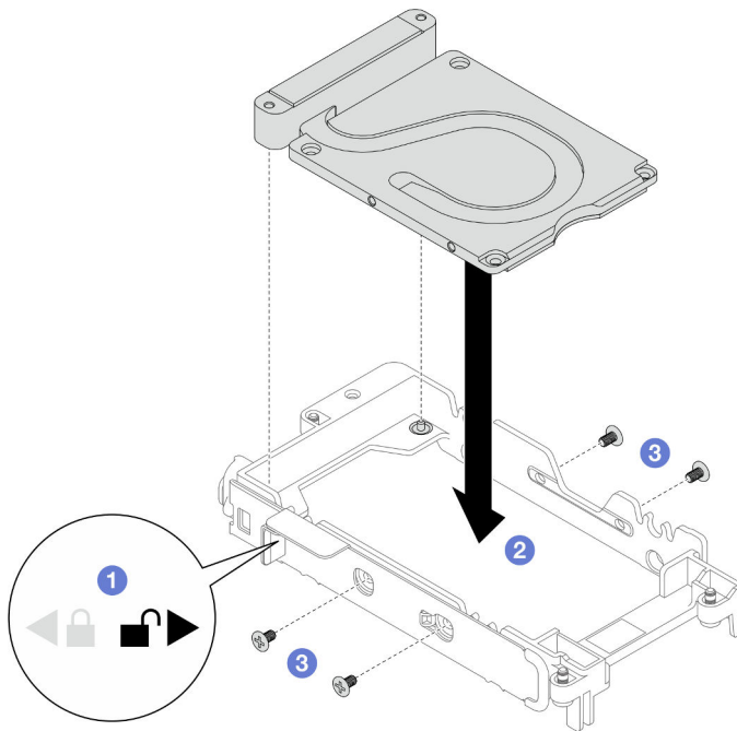
Abbildung 87. Installation der Leitplatte
