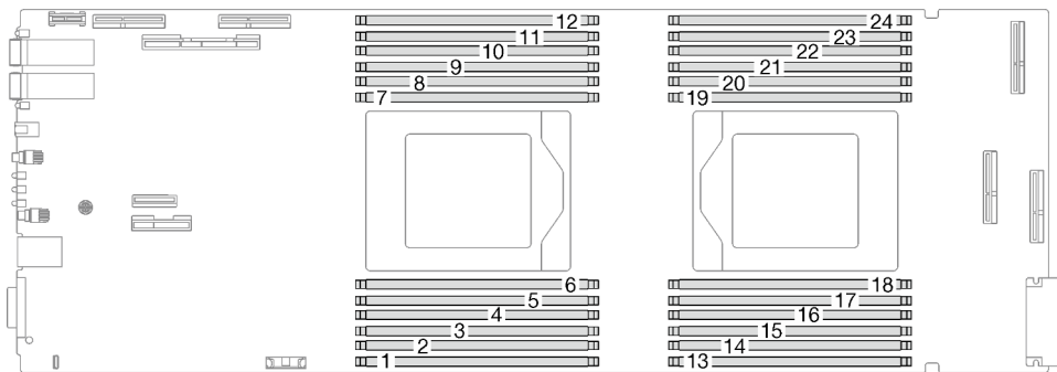
Abbildung 136. Position der Speichermodul-Anschlüsse
