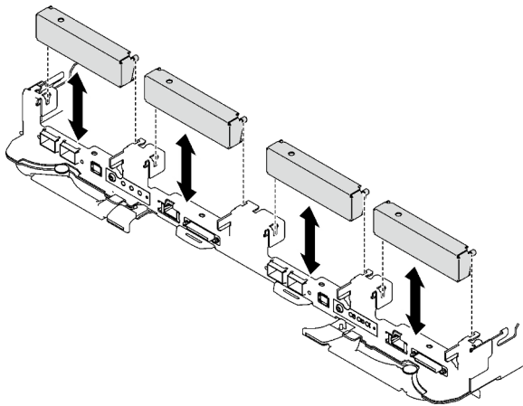
Abbildung 153. Installieren der Abdeckung der Frontblende
