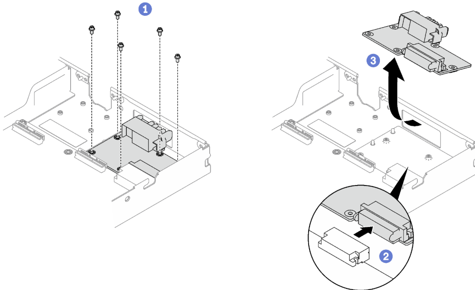
Abbildung 203. Entfernen der Stromversorgungsplatine
