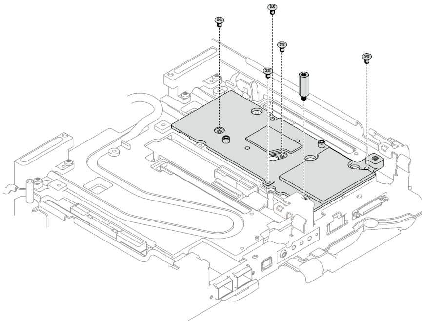
Abbildung 173. Installation der Schnittstellenplatte
