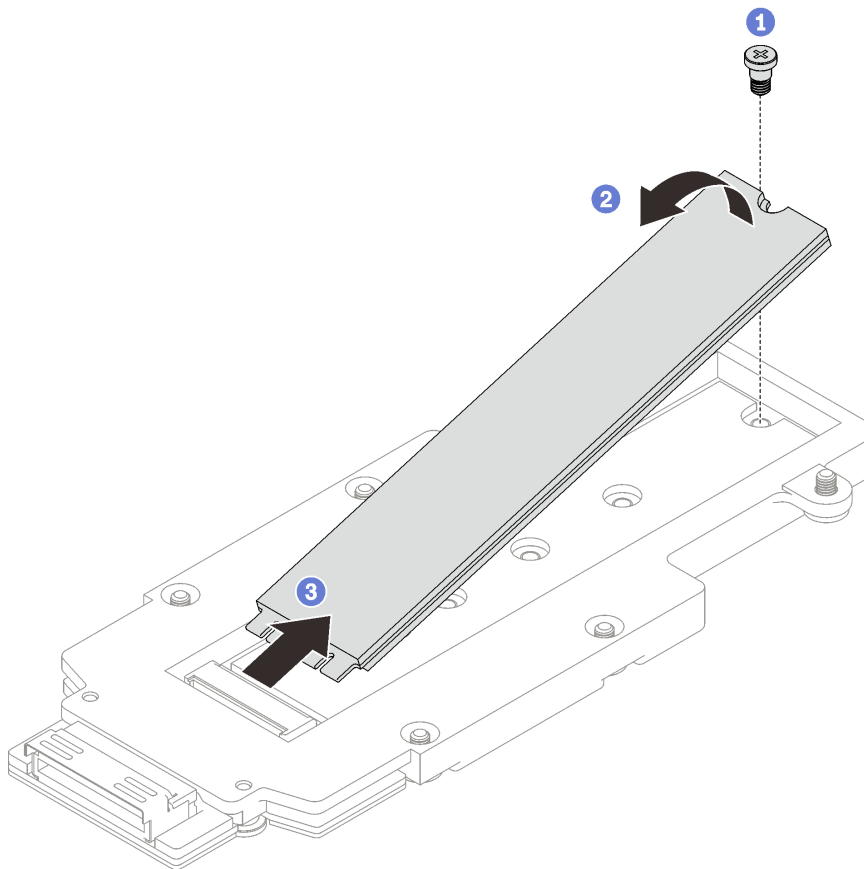
Abbildung 121. Entfernen des M.2-Laufwerks
