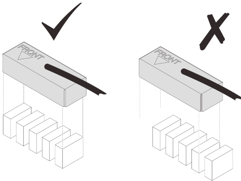
Abbildung 264. Abdeckung der Induktoren mit dem Abschirmrahmen
