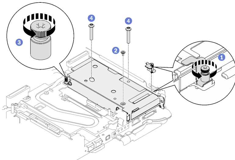
Abbildung 163. Lösen der PCIe-Adapterkartenbaugruppe von der Systemplatine
