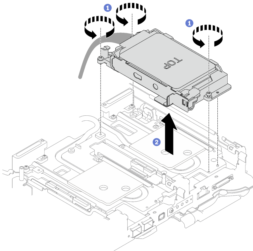
Abbildung 57. Entfernen der Laufwerkhalterung mit zwei 7-mm-Laufwerken
