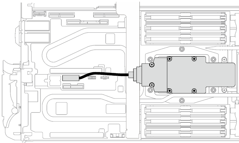
Abbildung 128. Installation des Kabels der M.2-Rückwandplattenbaugruppe
