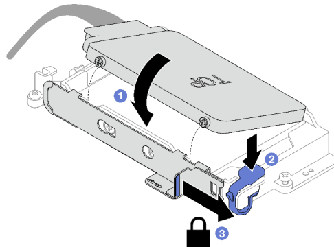
Abbildung 70. Installation des oberen Laufwerks
