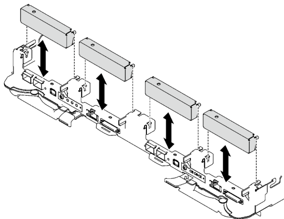
Abbildung 98. Entfernen der Abdeckblende für Frontblende
