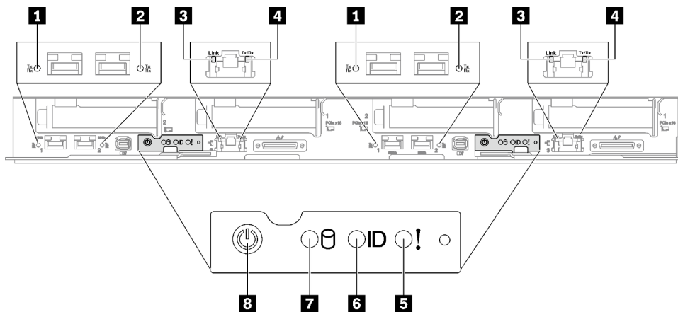
Abbildung 288. Anzeigen an der Vorderseite des SD665 V3 Einbaurahmens
