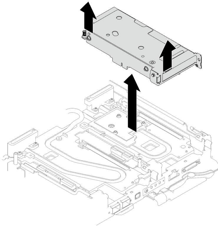
Abbildung 181. Entfernen der PCIe-Adapterrahmenbaugruppe
