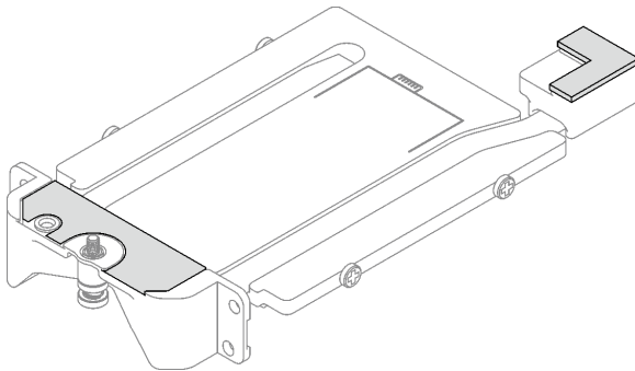
Abbildung 107. Austauschen der Putty-Pads der Leitplatte
