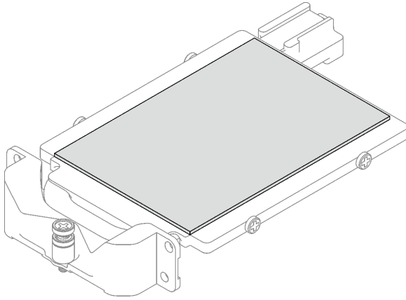
Abbildung 106. Austauschen des Gap-Pads der Leitplatte
