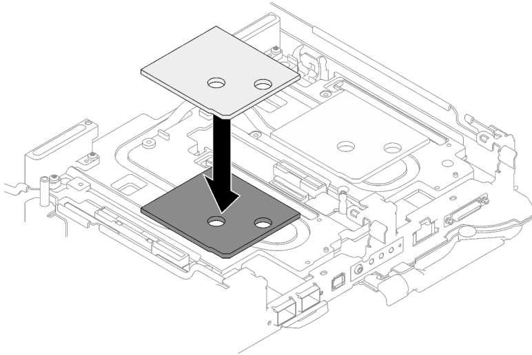
Abbildung 92. Austausch des Gap-Pads
