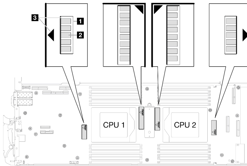
Abbildung 263. Induktorbefestigungspunkte
