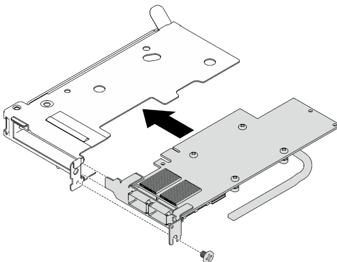
Abbildung 148. Installation des PCIe-Adapters
