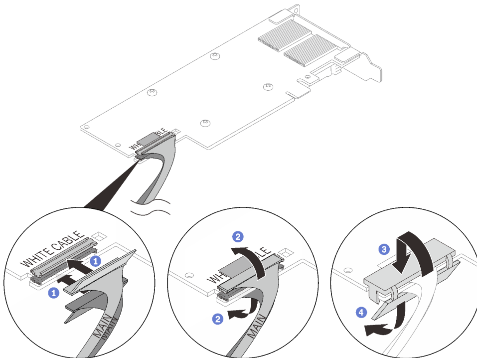
Abbildung 147. Installation des Kabels des PCIe-Adapters
