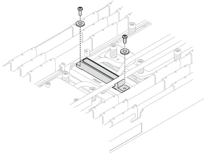
Abbildung 219. Schrauben der VR-Kühlplatte mit Unterlegscheiben
