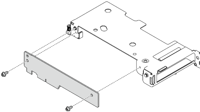
Abbildung 170. Entfernen der Erweiterungsplatine
