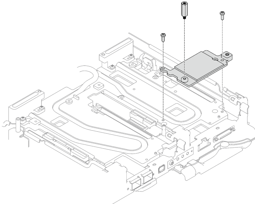
Abbildung 152. Entfernen der Schnittstellenplatte
