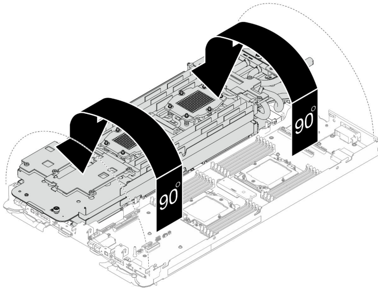
Abbildung 18. Wasserkreislauf falten
