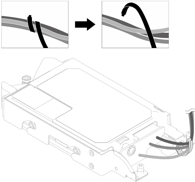
Abbildung 99. Lösen der Kabel aus dem Kabelbinder
