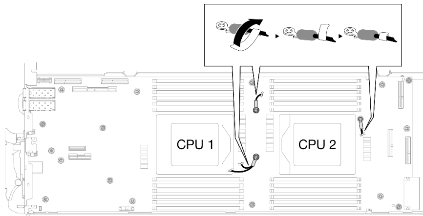
Abbildung 275. Rollen des Etiketts um das geschirmte Kabel
