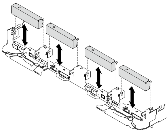
Abbildung 71. Installieren der Abdeckung der Frontblende
