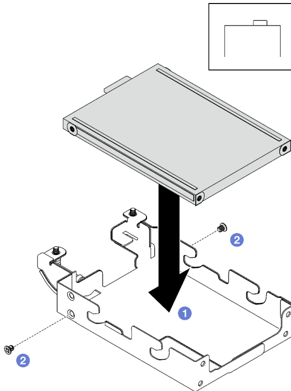
Abbildung 105. Installation des oberen E3.S-Laufwerks
