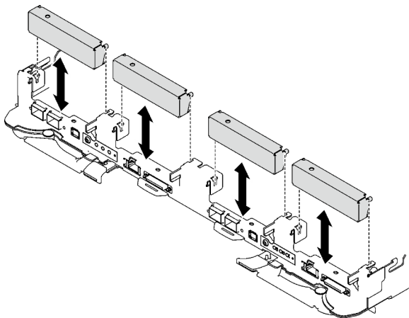
Abbildung 186. Installieren der Abdeckung der Frontblende
