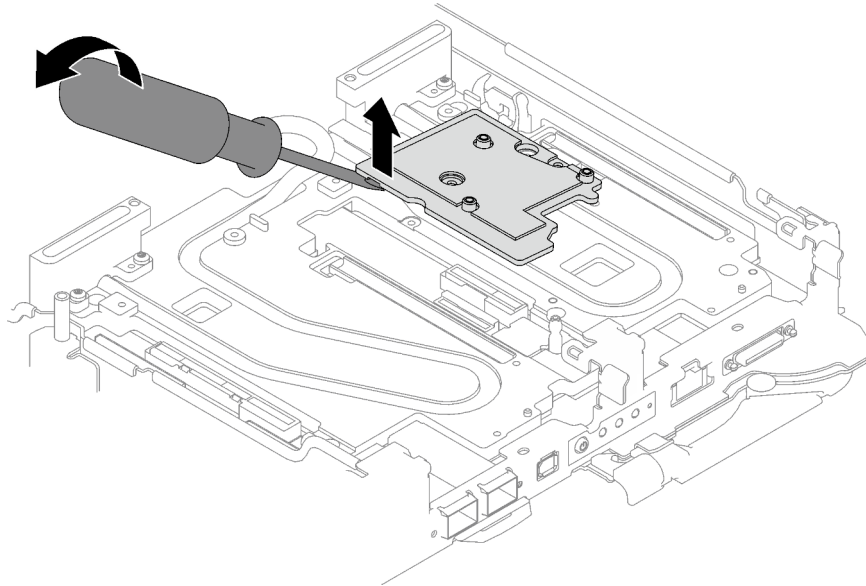
Abbildung 184. Lösen der Schnittstellenplatte von der Kühlplatte des Wasserkreislaufs
