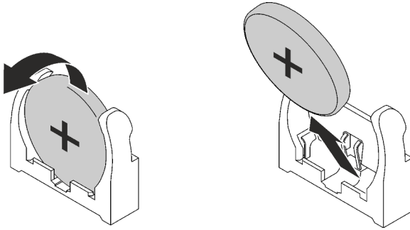
Abbildung 47. Entfernen der CMOS-Batterie
