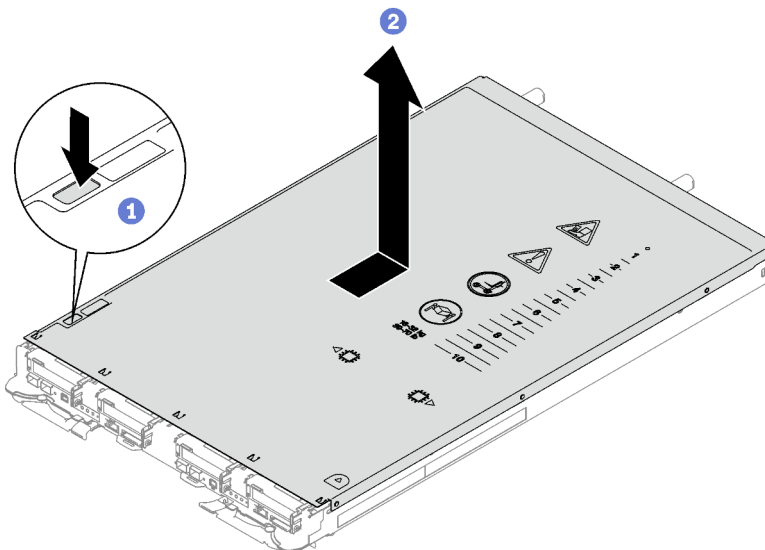
Abbildung 6. Entfernen der Abdeckung des Einbaurahmens
