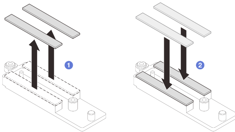
Abbildung 248. Austauschen der VR-Putty-Pads der Leiterplatte
