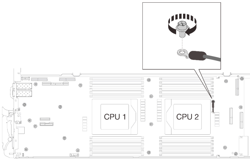
Abbildung 257. Installieren des geschirmten Kabels 4
