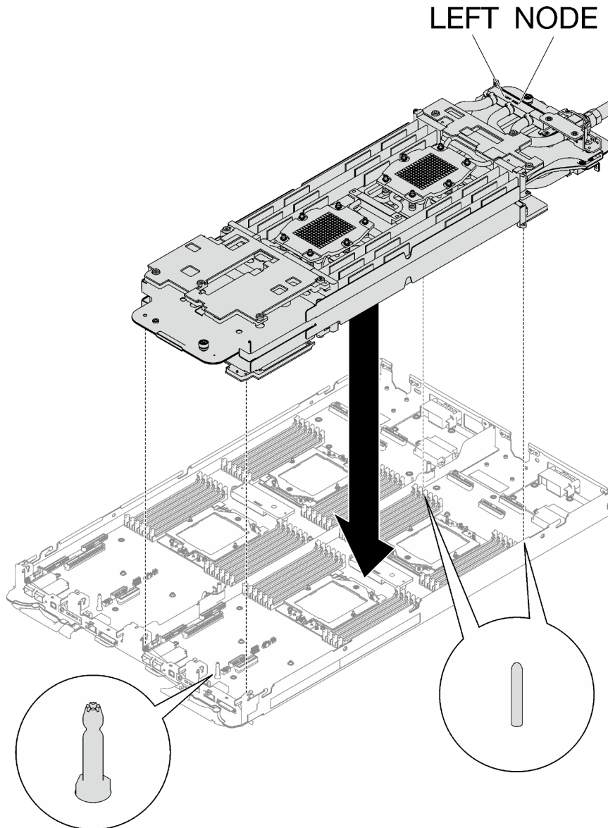
Abbildung 27. Installieren der Wasserkreislaufhalterung
