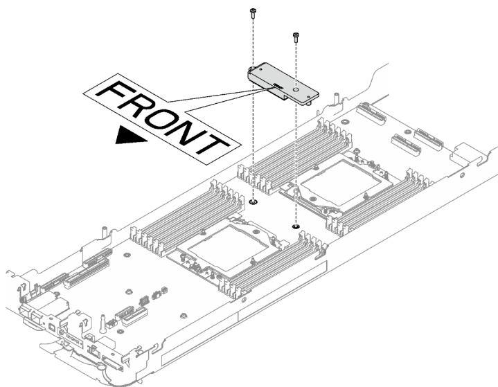
Abbildung 45. Entfernen der VR-Leitplatte
