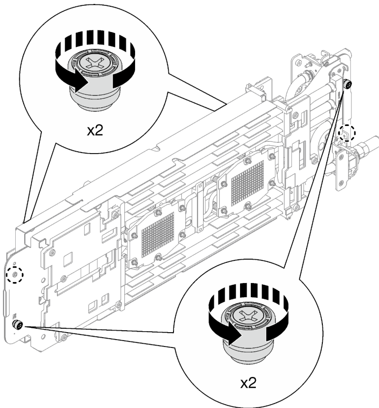
Abbildung 23. Lösen der unverlierbaren Rändelschrauben der Wasserkreislaufhalterung
