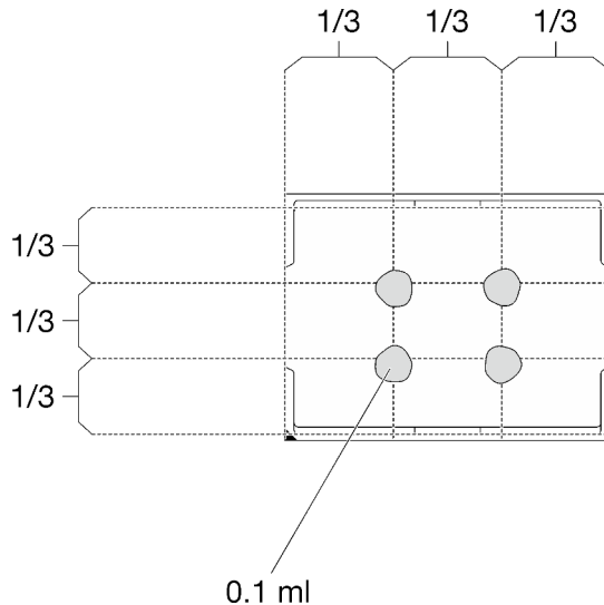
Abbildung 205. Auftragen der Wärmeleitpaste
