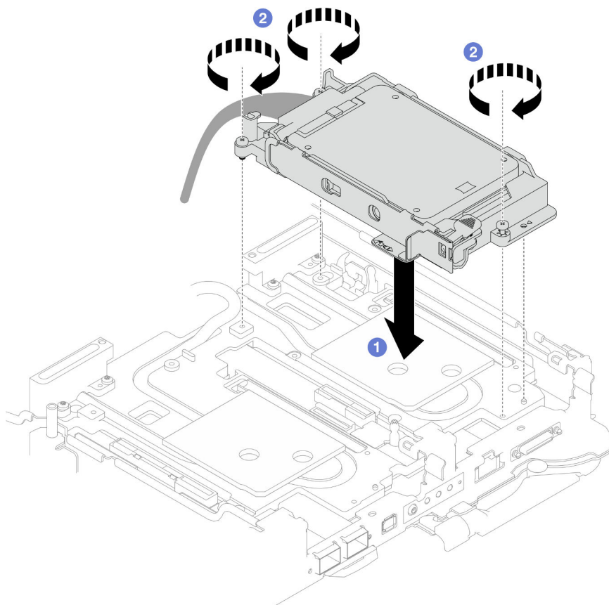
Abbildung 94. Installation einer 7-mm-NVMe-Laufwerkhalterungsbaugruppe
