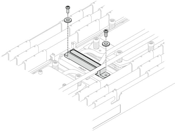
Abbildung 240. Schrauben der VR-Kühlplatte mit Unterlegscheiben
