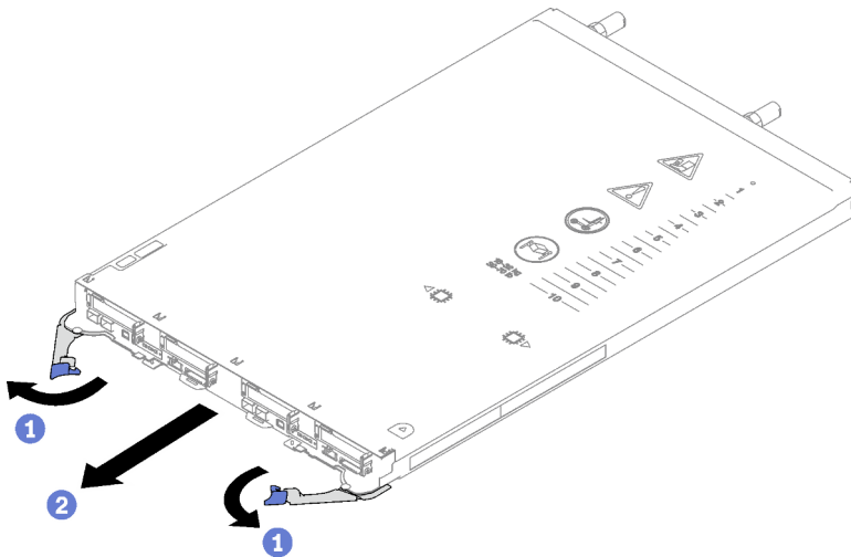
Abbildung 4. Einbaurahmen entfernen
