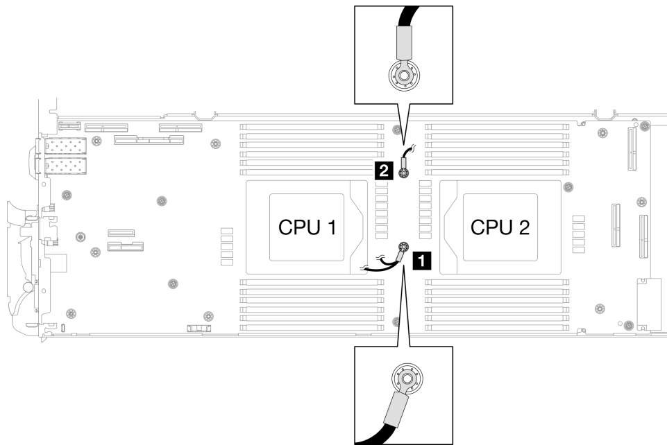
Abbildung 252. Ausrichten von abgeschirmtem Kabel 1/2 und abgeschirmtem Kabel 3 mit Schraubenlöchern
