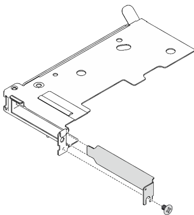
Abbildung 145. Installation der Abdeckblende
