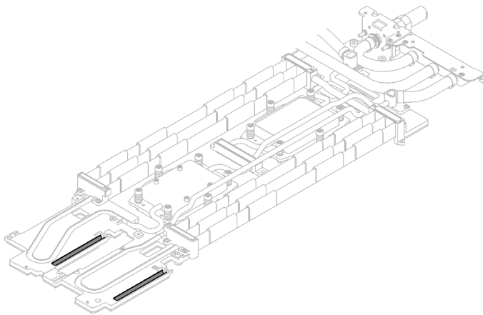
Abbildung 233. Gap-Pads am Wasserkreislauf (Oberseite)
