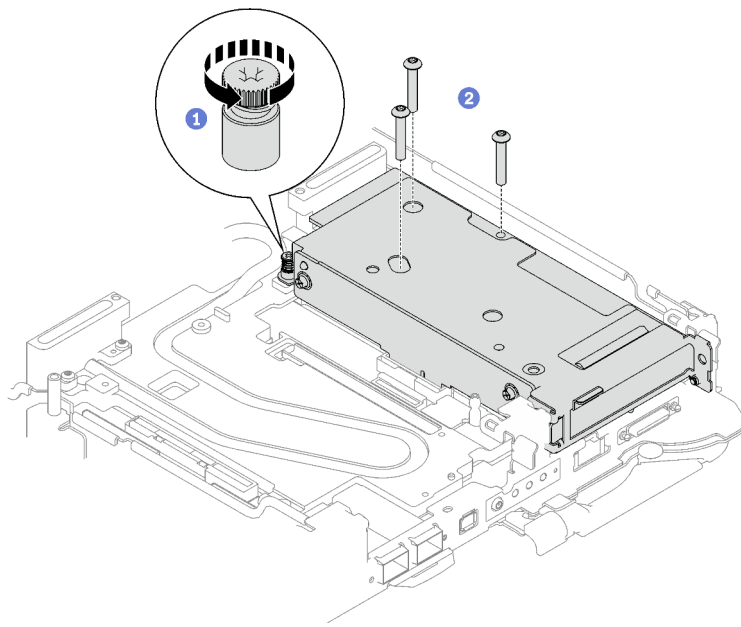
Abbildung 179. PCIe-Adapterkartenbaugruppe entfernen
