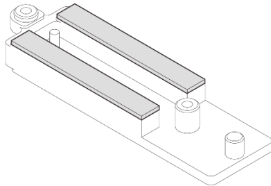
Abbildung 37. Putty-Pads an der Unterseite der VR-Leiterplatte
