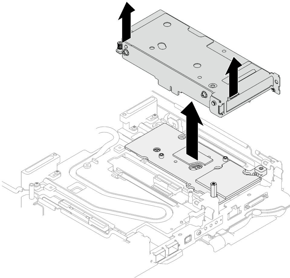
Abbildung 164. PCIe-Adapterkartenbaugruppe entfernen
