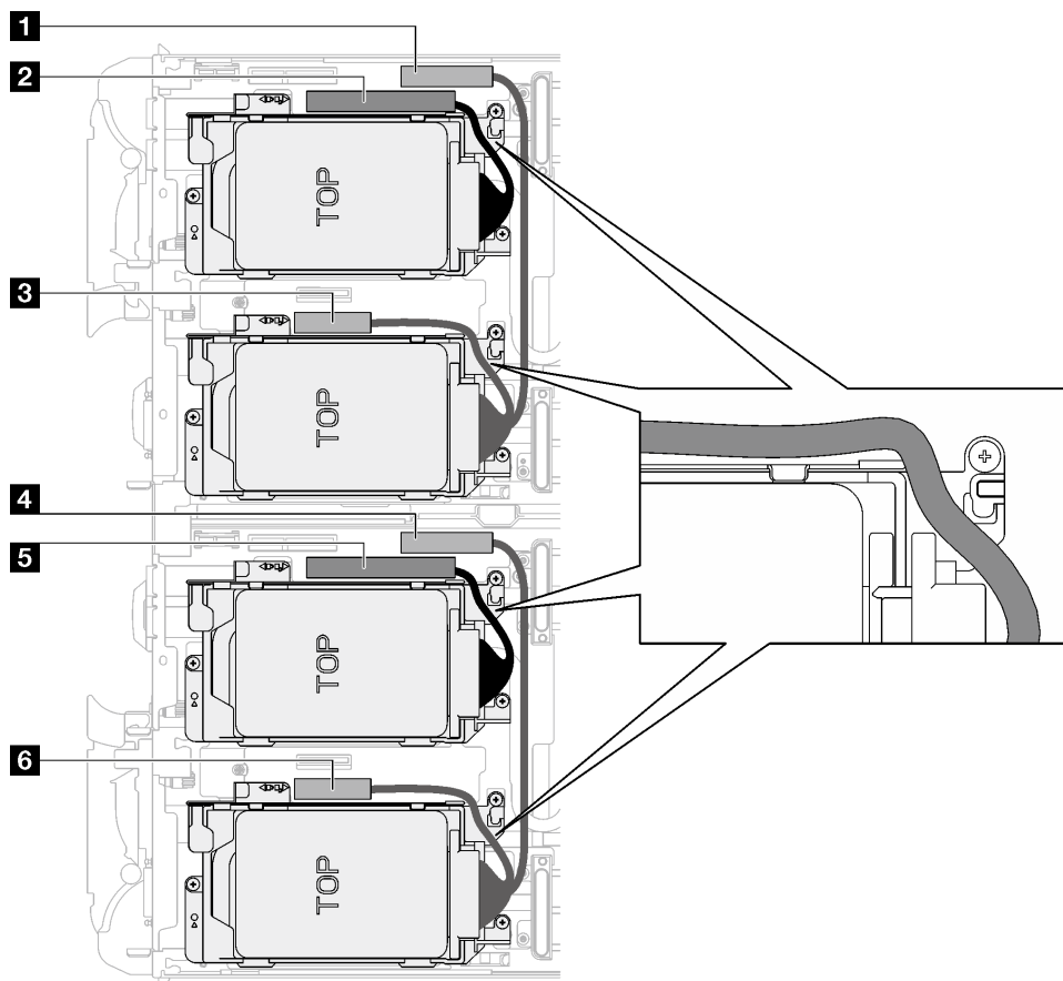
Abbildung 95. Kabelführung der Laufwerkbaugruppe für alle NVMe-Laufwerke
