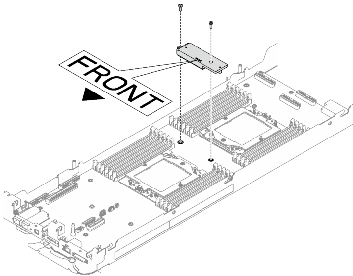
Abbildung 244. Entfernen der VR-Leitplatte
