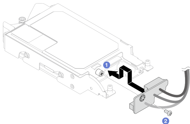
Abbildung 110. Installation der kabelgebundenen E3.S-Rückwandplatine
