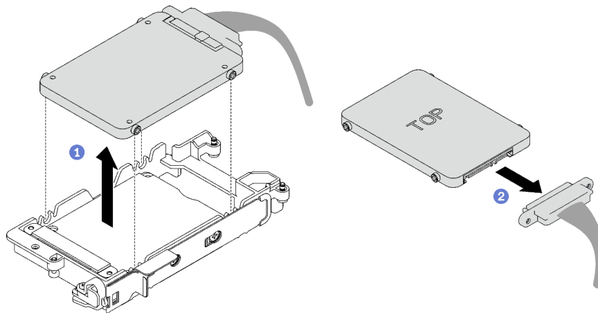
Abbildung 63. Entfernen des unteren Laufwerks
