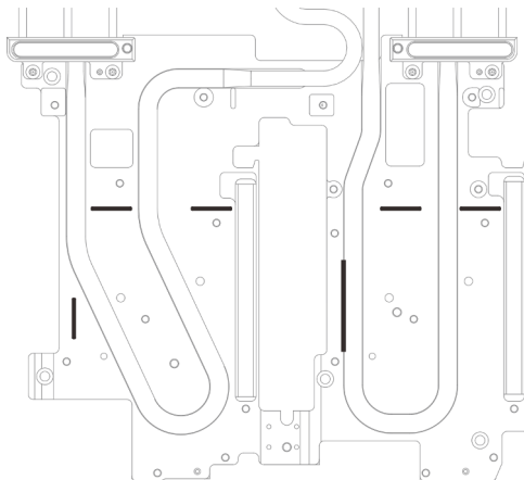
Abbildung 91. Markierungen auf dem Wasserkreislauf für die Ausrichtung des Gap Pad
