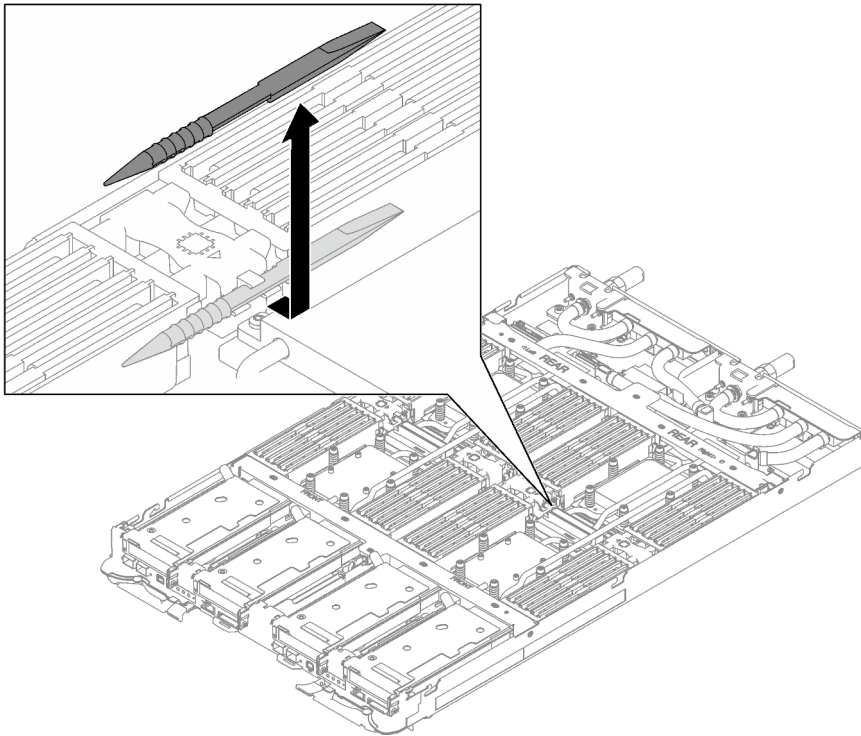
Abbildung 137. Entfernen des Speichermodul-Werkzeugs
