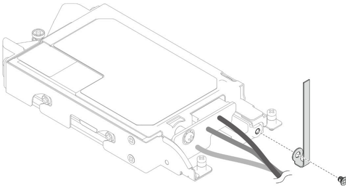
Abbildung 100. Entfernen des Kabelbinders
