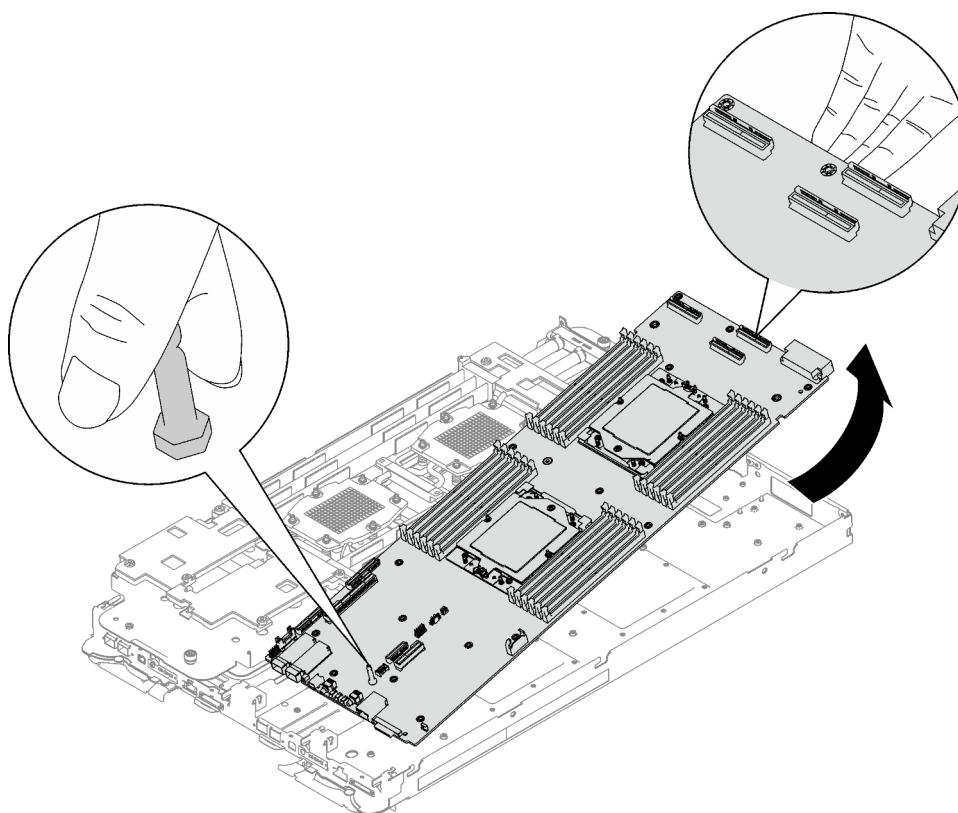
Abbildung 246. Entfernen der Systemplatine
