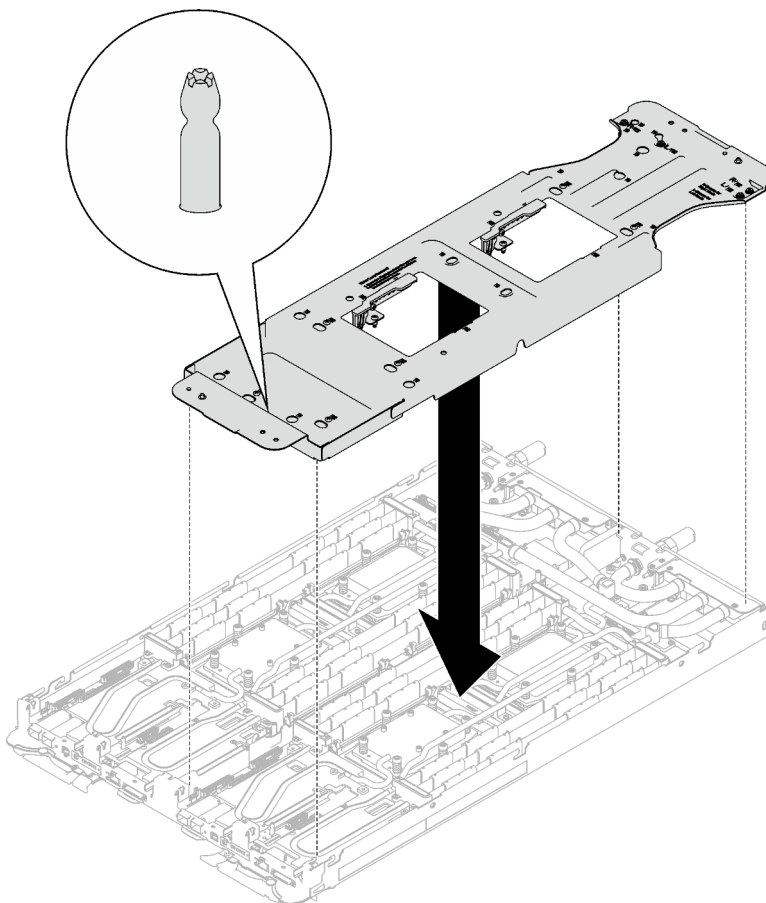
Abbildung 197. Installieren der Wasserkreislaufhalterung
