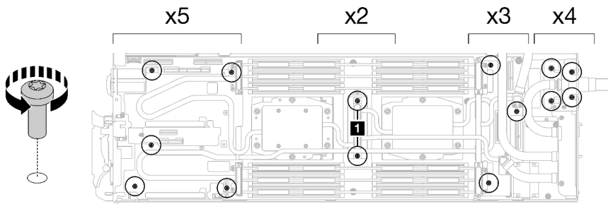
Abbildung 196. Entfernen der Schrauben des Wasserkreislaufs
