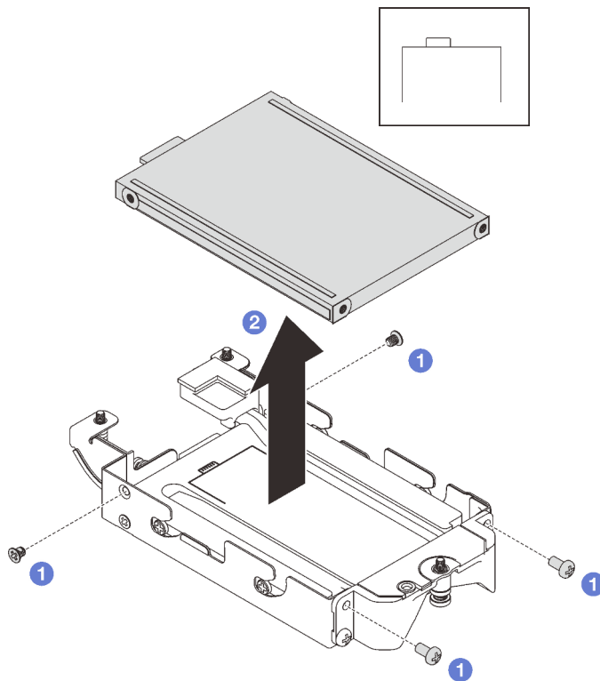
Abbildung 102. Entfernen des unteren E3.S-Laufwerks
