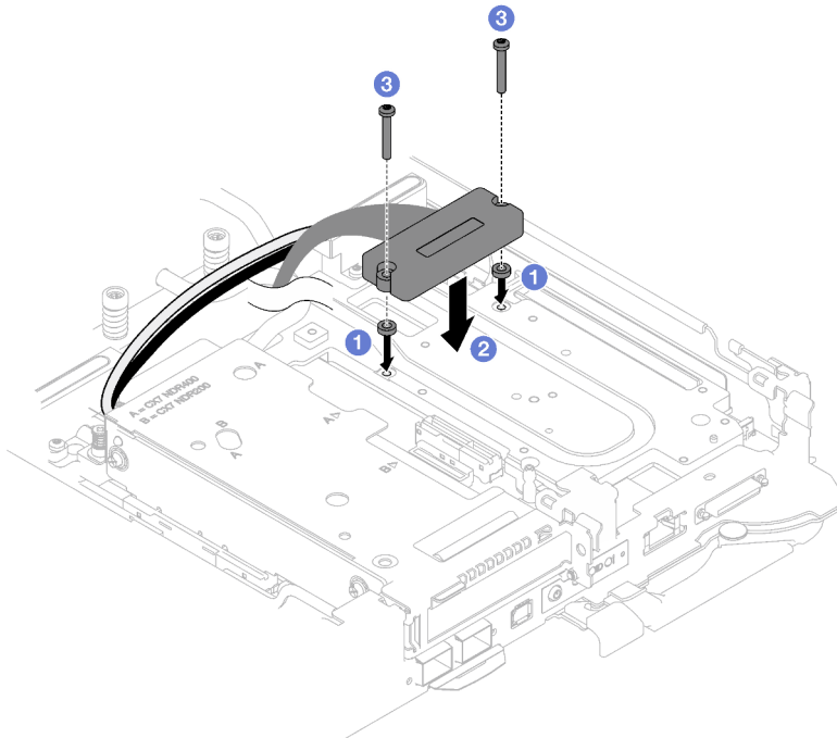
Abbildung 193. Verbindungskabel installieren
