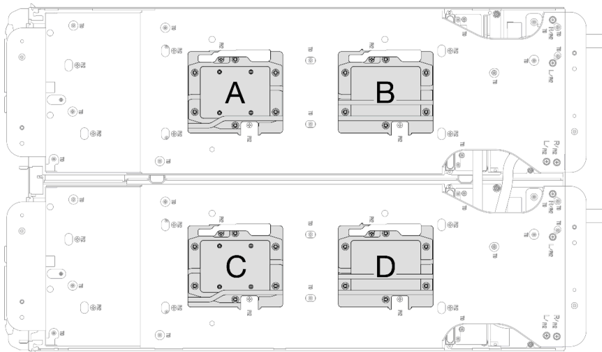
Abbildung 211. Installieren der Prozessorkühlplatte
