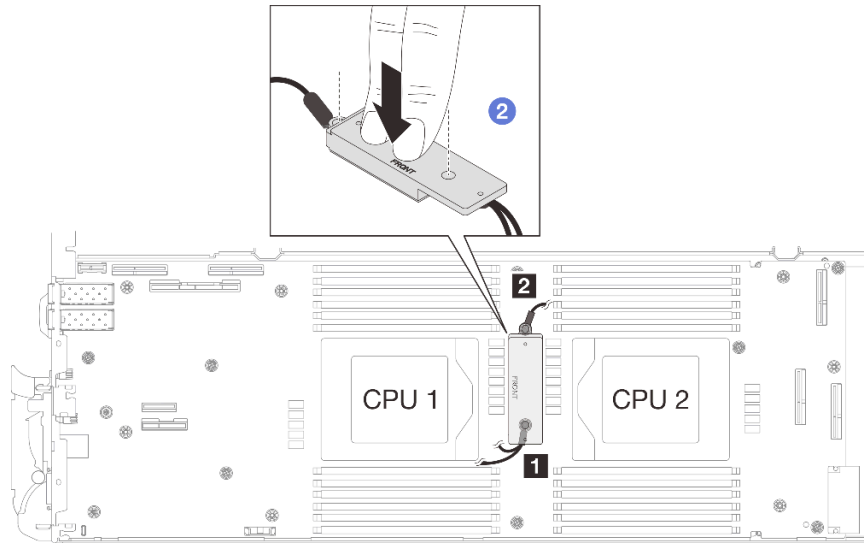
Abbildung 254. Drücken auf die VR-Leiterplatte
