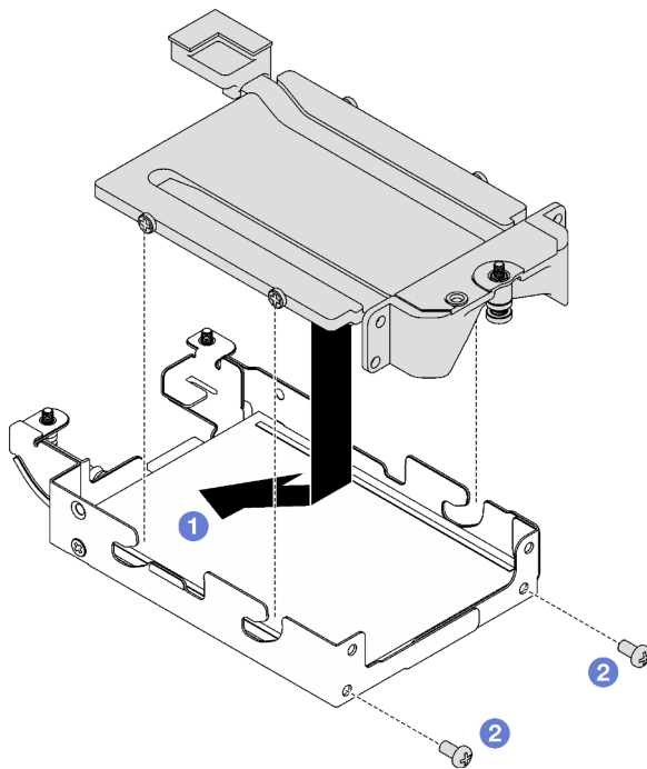
Abbildung 108. Installation der Leitplatte für E3.S-Laufwerk
