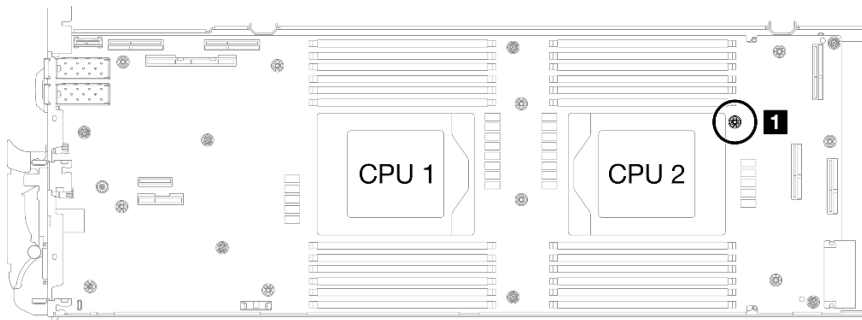
Abbildung 256. Position des Schraubenlochs von geschirmtem Kabel 4
