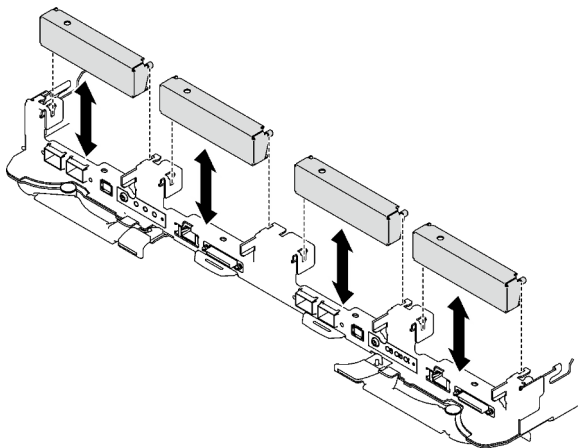
Abbildung 169. Installieren der Abdeckung der Frontblende
