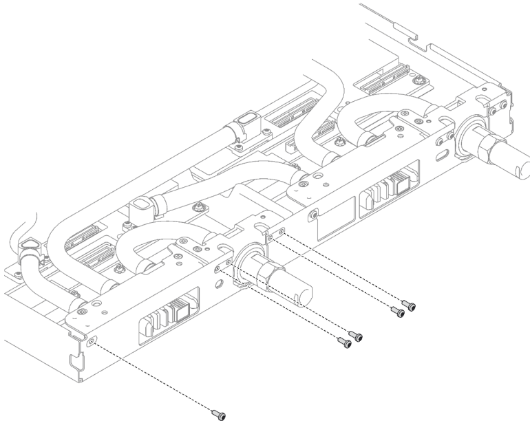
Abbildung 194. Entfernen der Schrauben vom Schnellanschluss
