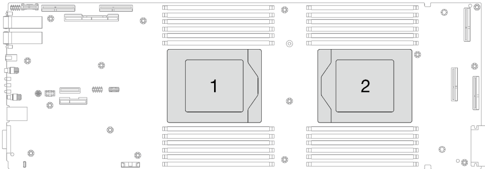
Abbildung 228. Positionen der Prozessoren
