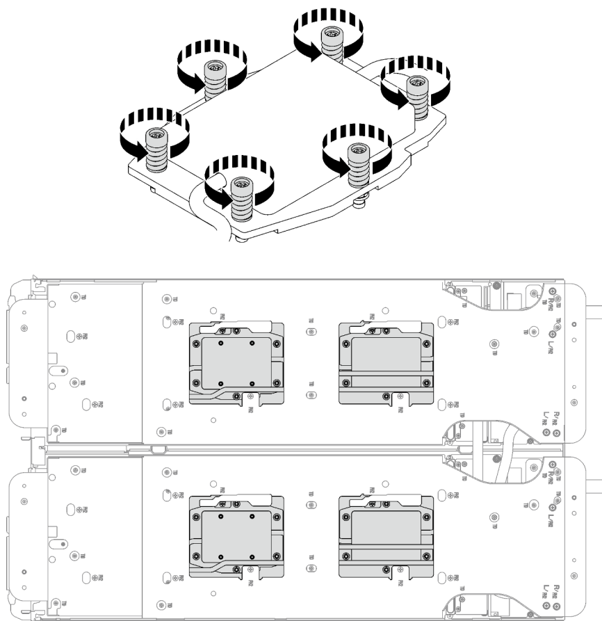
Abbildung 224. Entfernen der Prozessorkühlplatte
