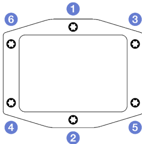
Abbildung 199. Etikett an der Prozessorkühlplatte
