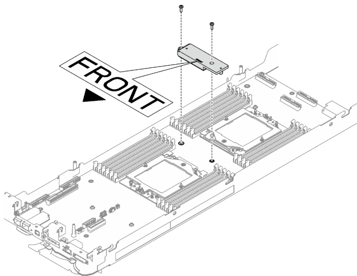
Abbildung 279. Installation der VR-Leitplatte
