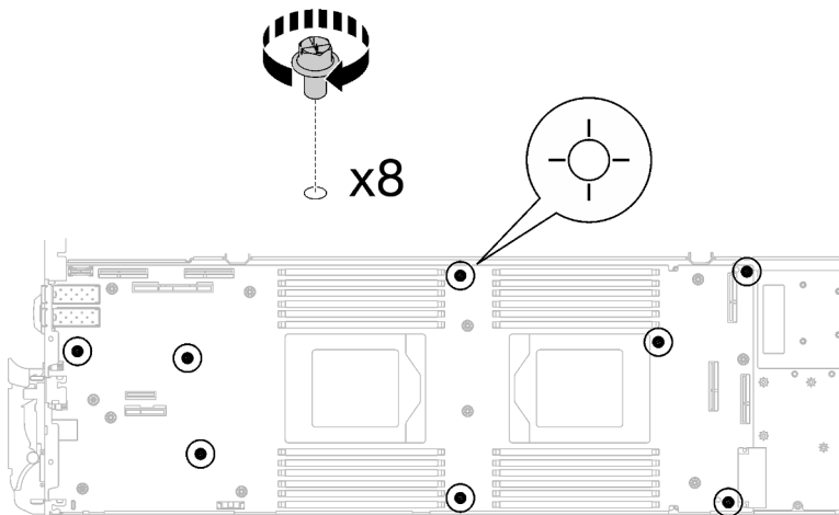
Abbildung 245. Entfernen der Schrauben der Systemplatine
