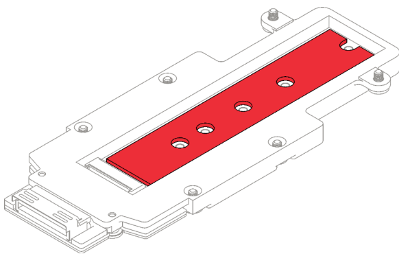
Abbildung 122. Gap-Pad auf der M.2-Rückwandplatine
