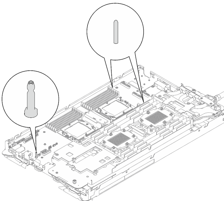
Abbildung 28. Führungsstifte an der linken Seite des Rechenknotens
