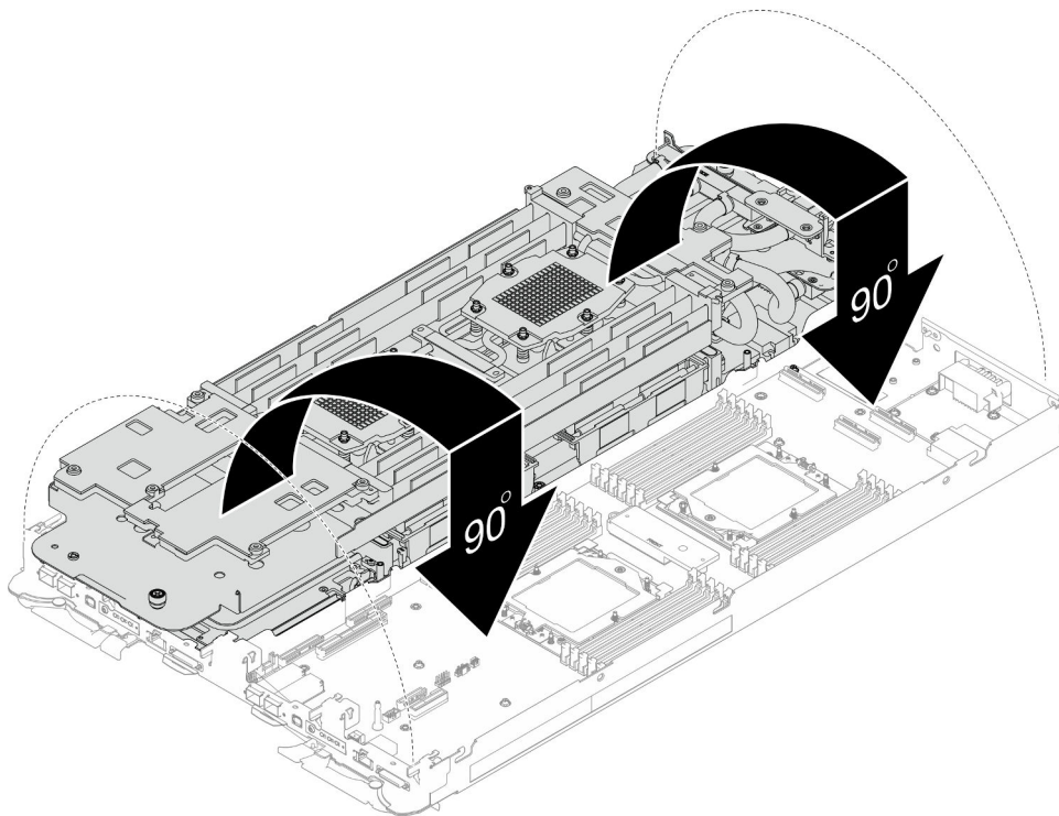
Abbildung 210. Installieren des Wasserkreislaufs
