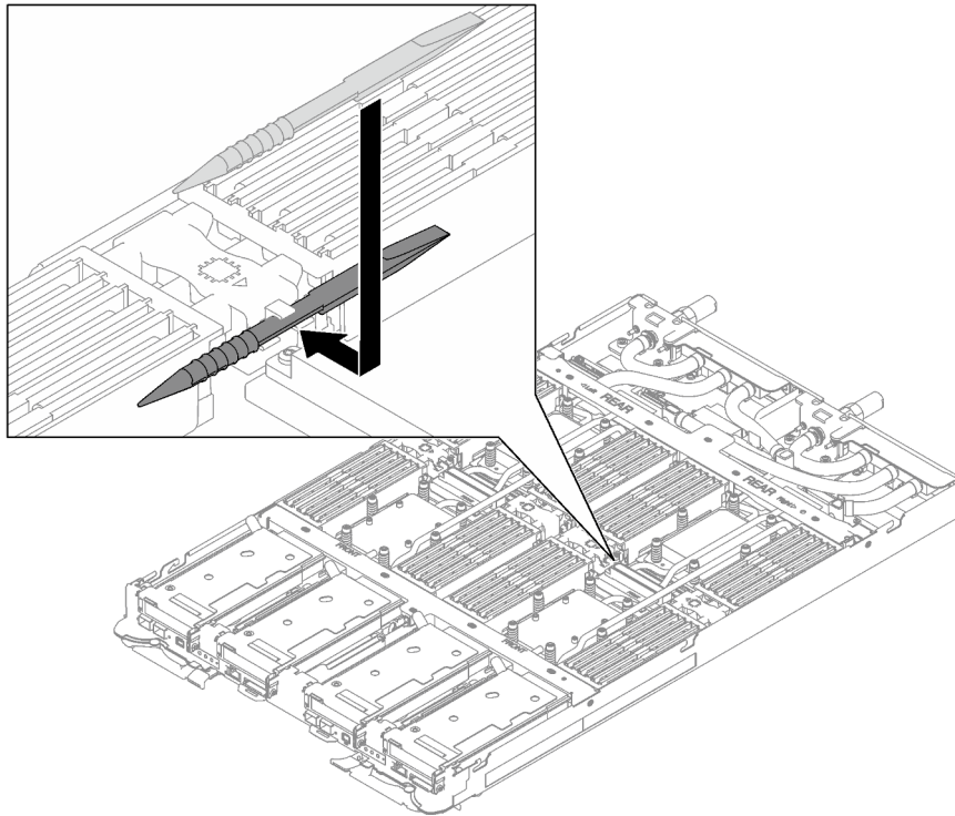
Abbildung 53. Befestigen des Speichermodul-Werkzeugs
