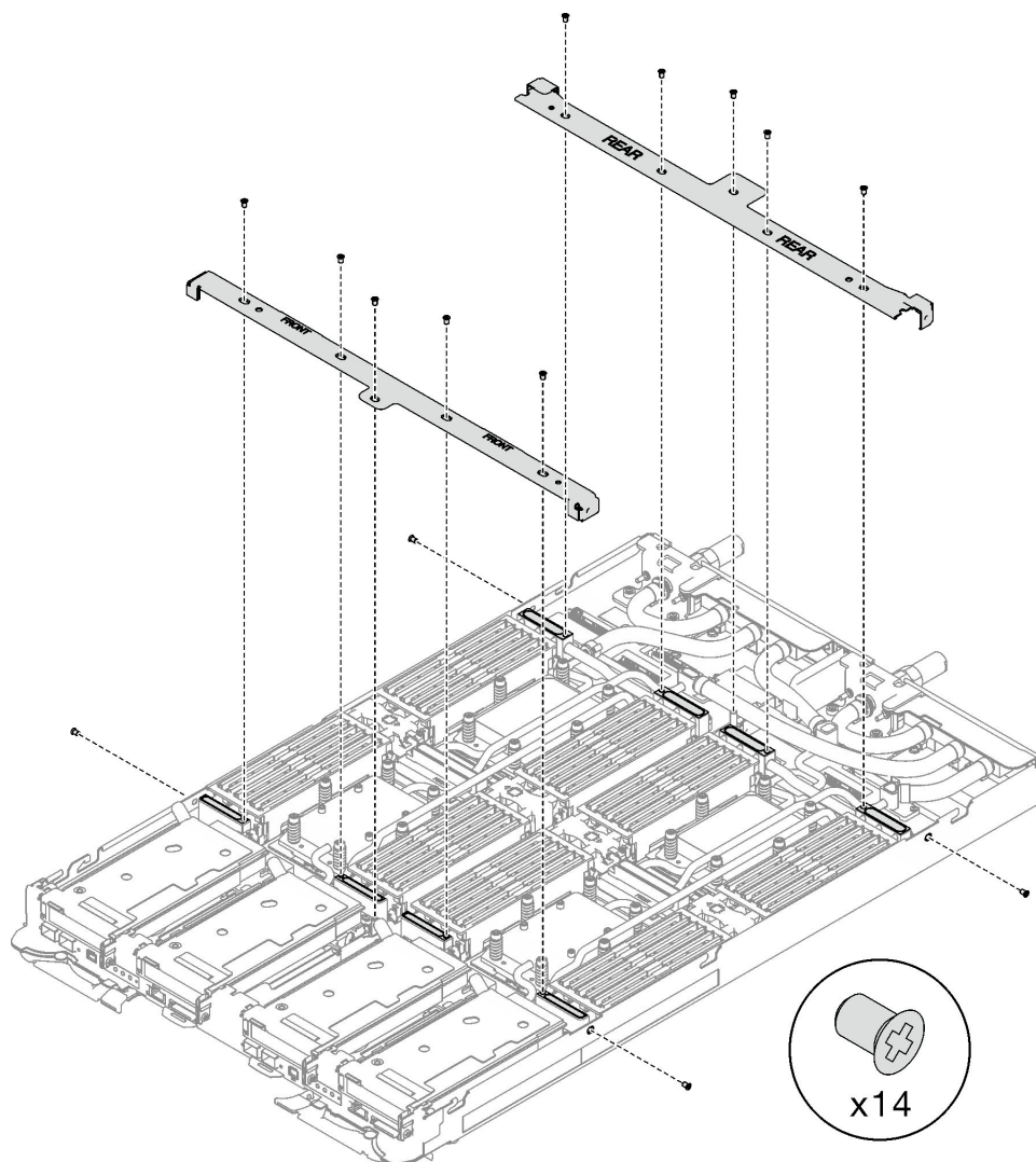
Abbildung 9. Querstreben installieren
