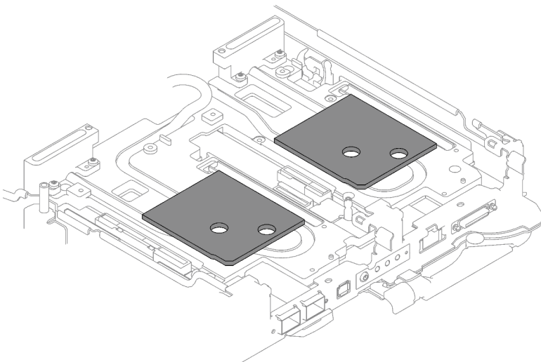
Abbildung 75. Positionen der Gap-Pads
