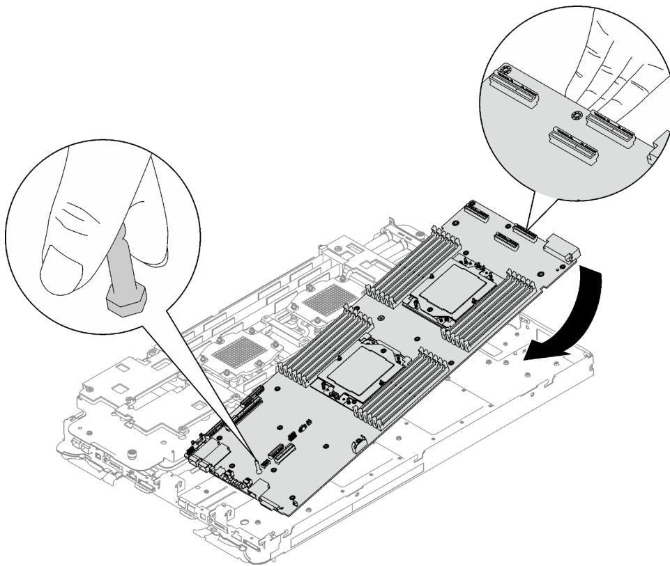
Abbildung 269. Systemplatineinbau
