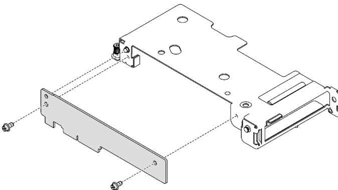
Abbildung 187. Entfernen der Erweiterungsplatine
