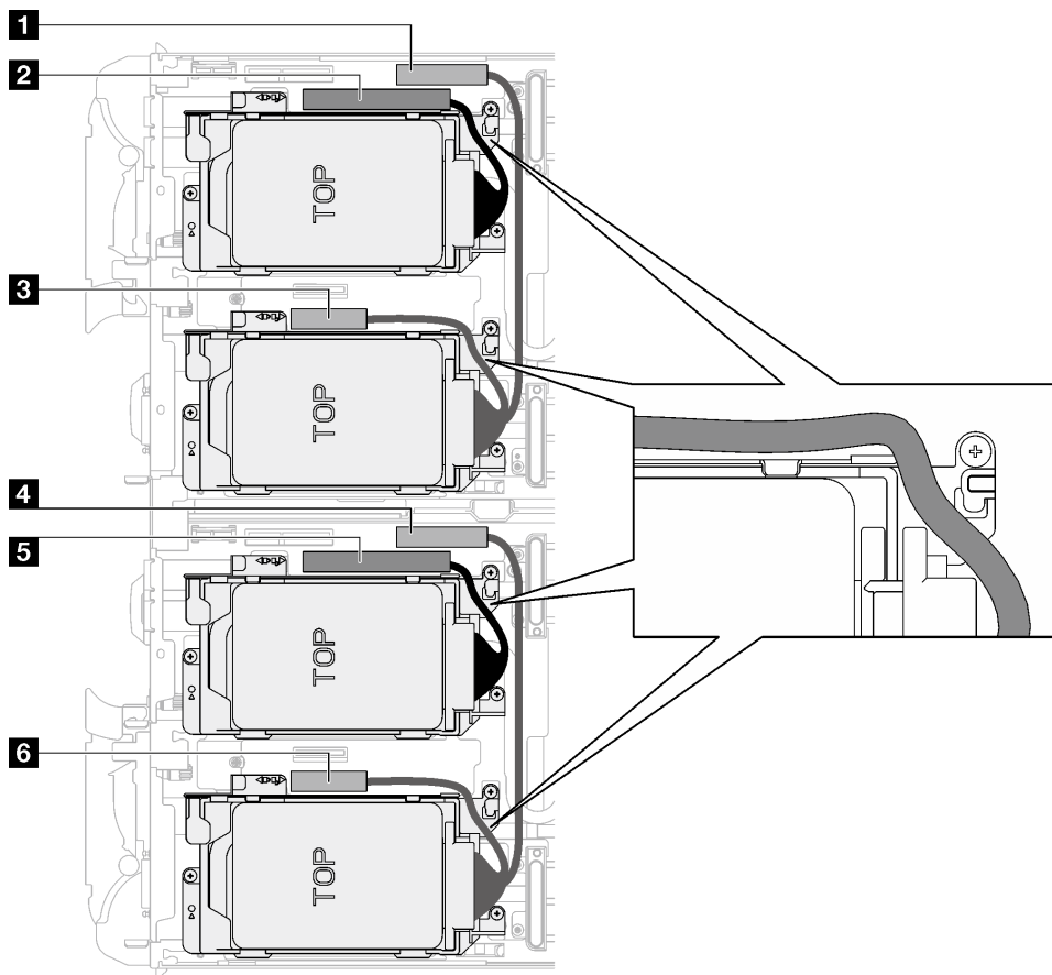
Abbildung 55. Kabelführung der Laufwerkbaugruppe für alle NVMe-Laufwerke
