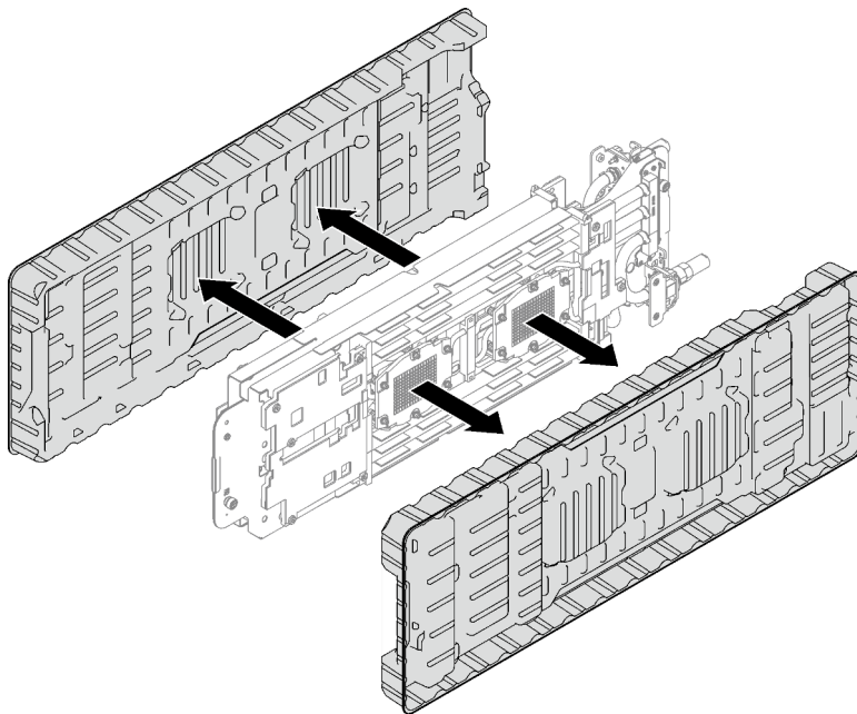
Abbildung 231. Entfernen der Kunststoffabdeckungen der Wärmeleitpaste
