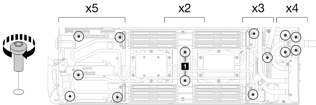
Abbildung 34. Installieren der Schrauben am Wasserkreislauf und Schnellanschluss
