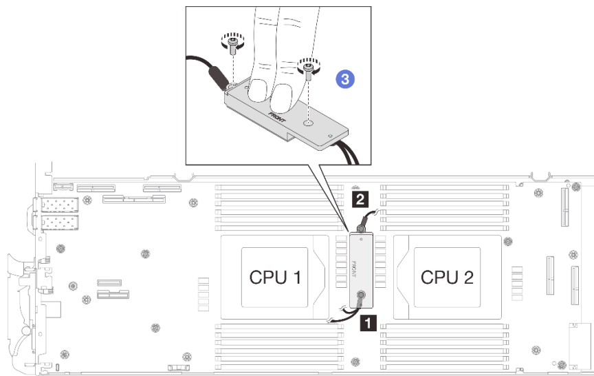
Abbildung 272. Installieren der geschirmten Kabel 1/2 und 3
