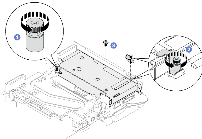
Abbildung 150. Entfernen der unverlierbaren Schraube der Klemmbefestigung
