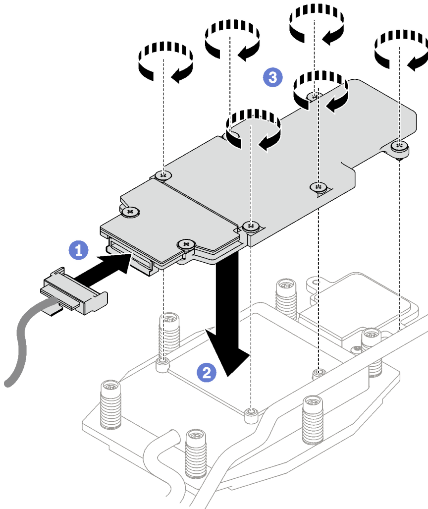
Abbildung 127. Installation der M.2-Rückwandplattenbaugruppe
