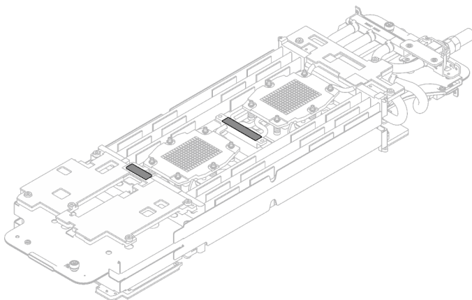
Abbildung 26. Putty-Pads am Wasserkreislauf
