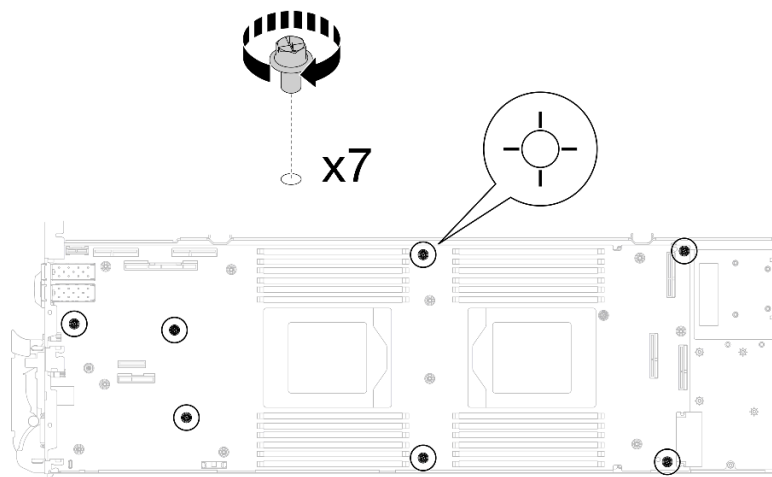
Abbildung 266. Anbringen der Systemplatinenschrauben
