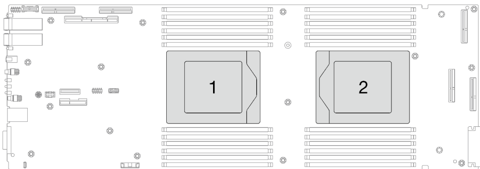
Abbildung 217. Positionen der Prozessoren
