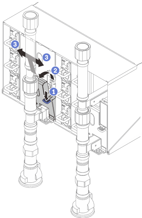
Abbildung 295. Entfernen der unteren EMV-Abschirmung
