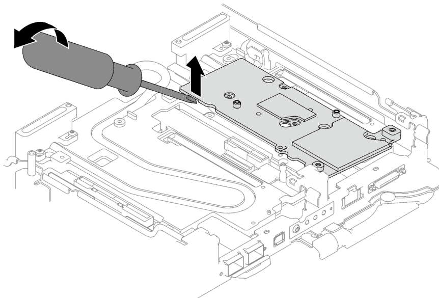
Abbildung 167. Lösen der Schnittstellenplatte von der Kühlplatte des Wasserkreislaufs
