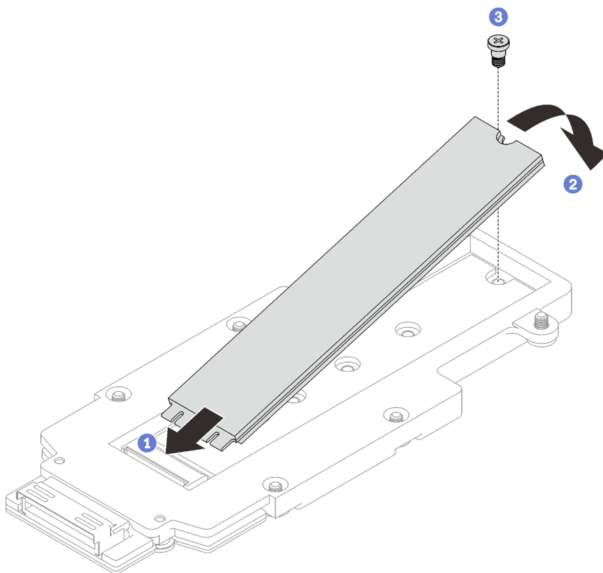
Abbildung 123. Installieren des M.2-Laufwerks
