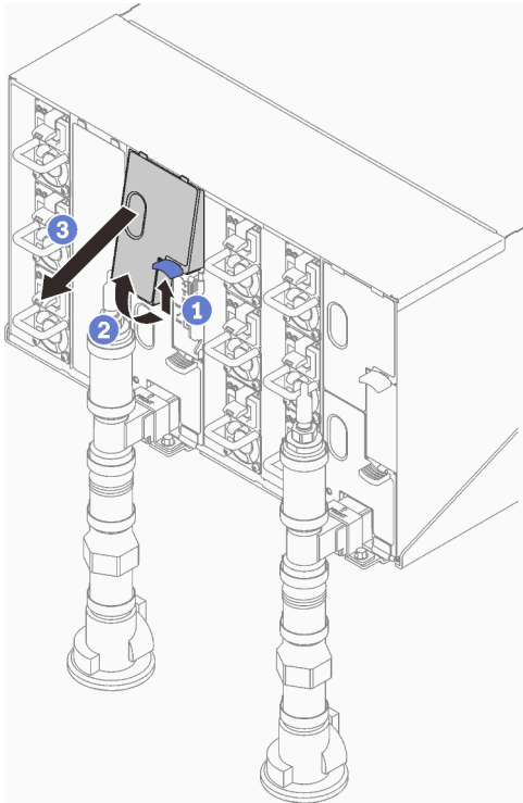
Abbildung 296. Entfernen der oberen EMV-Abschirmung
