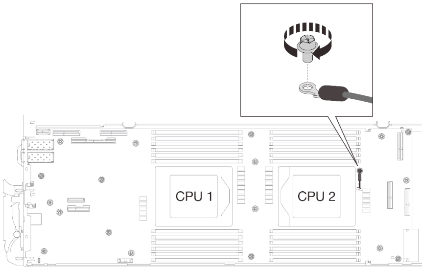
Abbildung 274. Installieren des geschirmten Kabels 4
