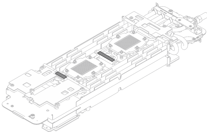
Abbildung 234. Putty-Pads am Wasserkreislauf
