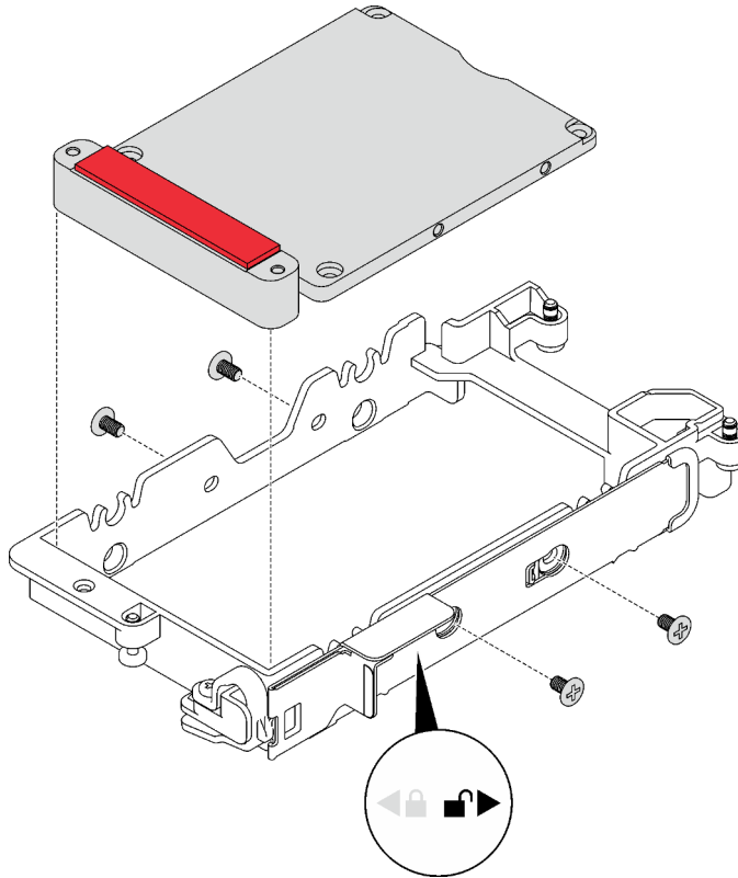
Abbildung 68. Installation der Leitplatte
