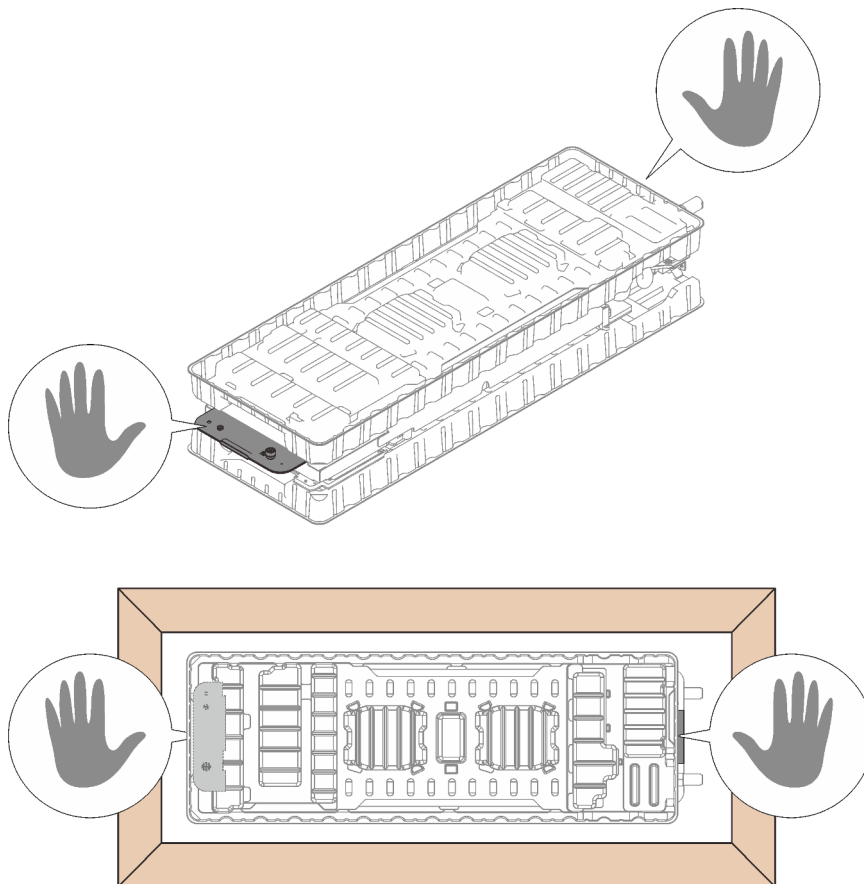
Abbildung 21. Berührungspunkte bei der Entnahme des Wasserkreislaufs aus der Verpackung
