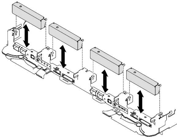
Abbildung 113. Installieren der Abdeckung der Frontblende
