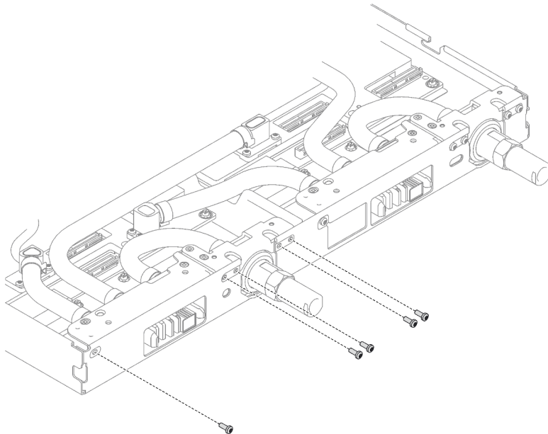
Abbildung 218. Entfernen der Schrauben vom Schnellanschluss
