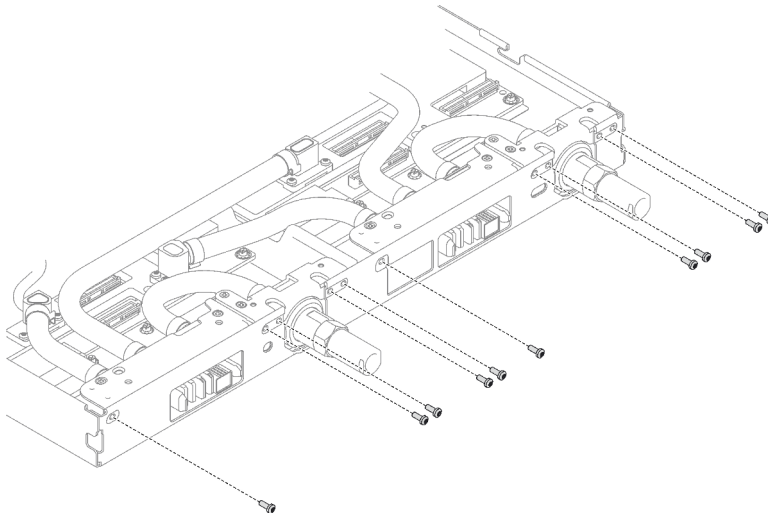
Abbildung 10. Entfernen der Schrauben vom Schnellanschluss
