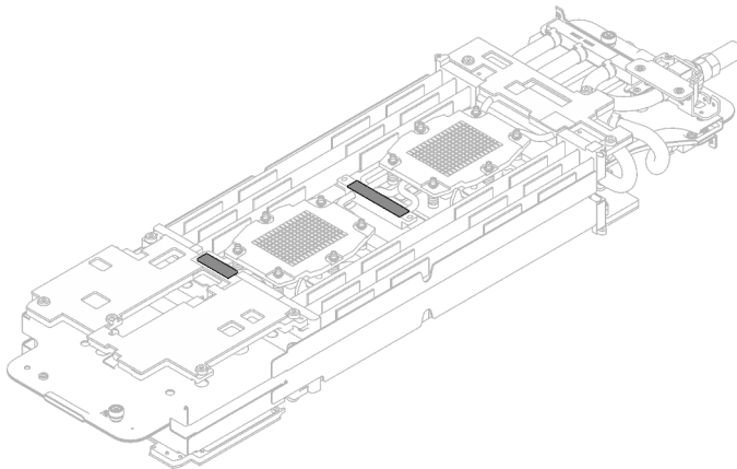
Abbildung 208. Putty-Pads am Wasserkreislauf
