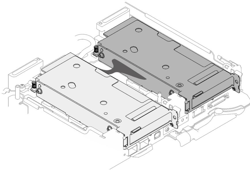
Abbildung 188. Typen von PCIe-Adapterkarten, die in Steckplatz 1 und Steckplatz 2 installiert sind
