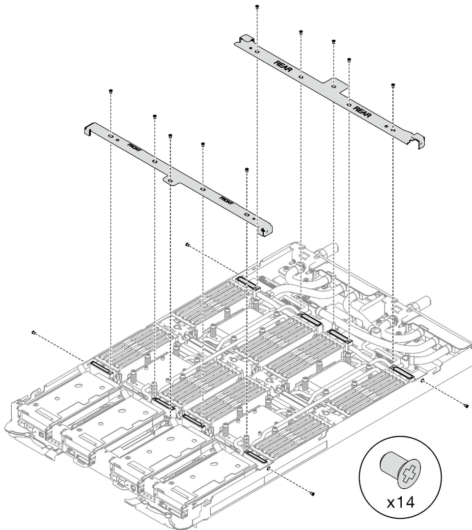
Abbildung 8. Entfernen der Querstrebe
