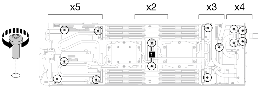
Abbildung 220. Entfernen der Schrauben des Wasserkreislaufs
