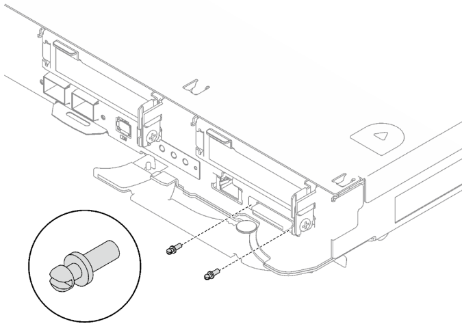
Abbildung 277. Anbringen der KVM-Schrauben
