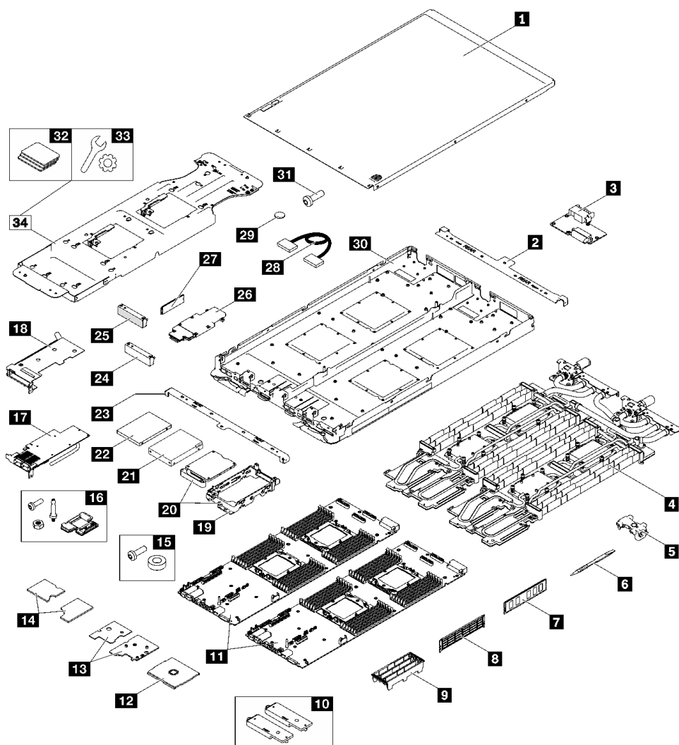
図 14. SD665 V3 部品リスト
