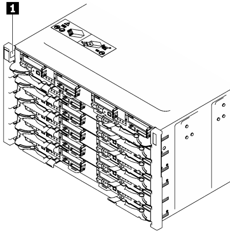
図 15. エンクロージャー前面のエンクロージャー・ラベル
