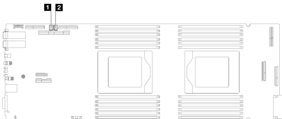
図6. 計算ノードのシステム・ボード上にあるスイッチ
