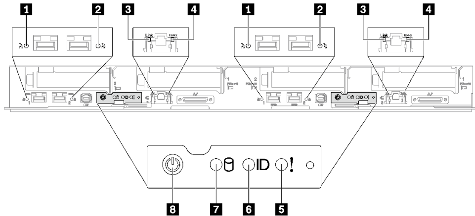
図8. SD665 V3 トレイの前面 LED
