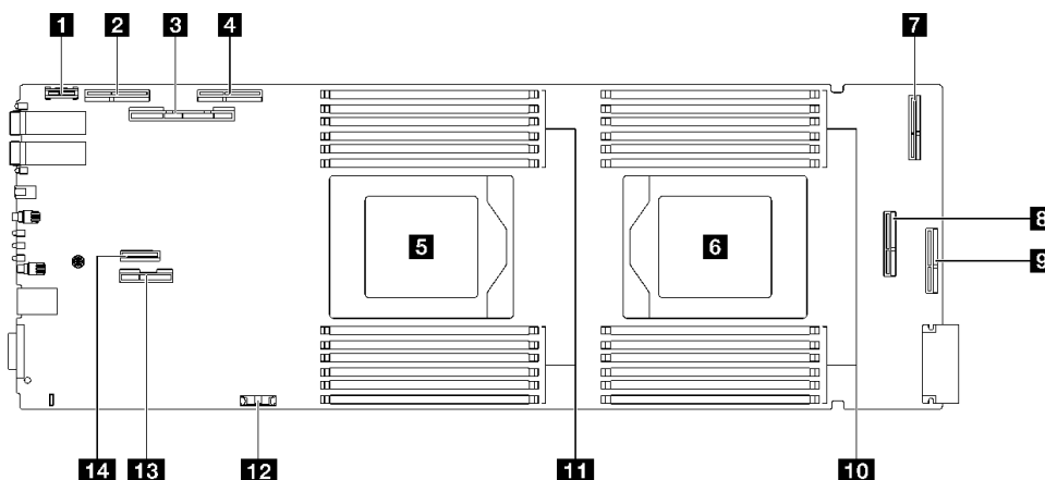
図5. 計算ノード・システム・ボード上の内部コネクタ
