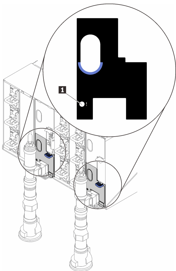
図 12. ドリップ・センサー LED
