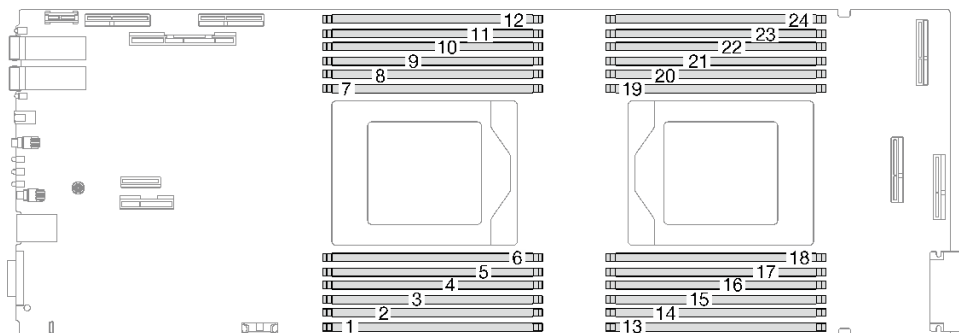
図4. 計算ノード・システム・ボード上の DIMM スロット番号
