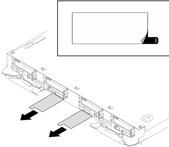
図 17. 引き出し式情報タブにある Lenovo XClarity Controller のネットワーク・アクセス・ラベル
