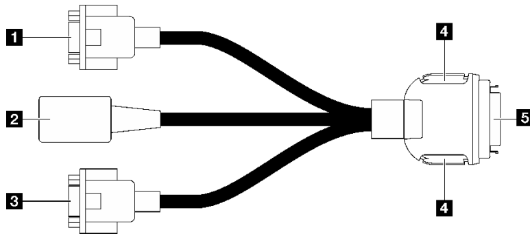
図 3. KVM ブレークアウト・ケーブルのコネクタおよびコンポーネント
