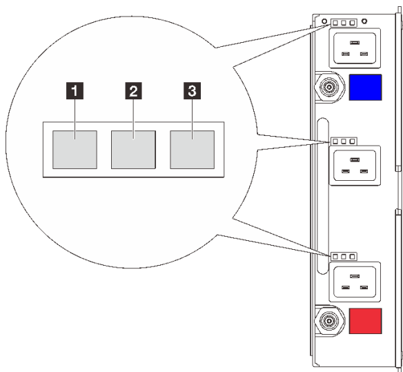
図 11. DWC パワー・サプライ LED
