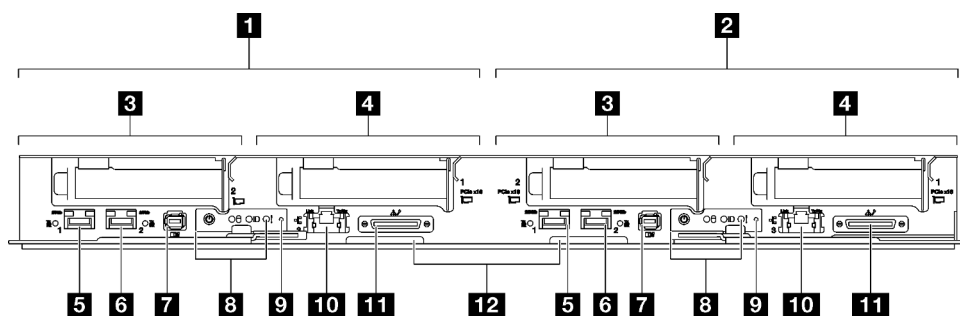
図 1. SD665 V3 トレイ
