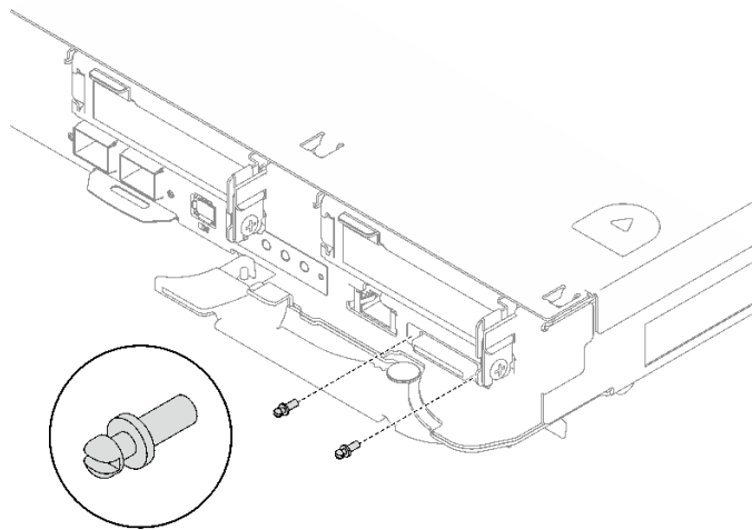
그림 281. KVM 나사 설치
