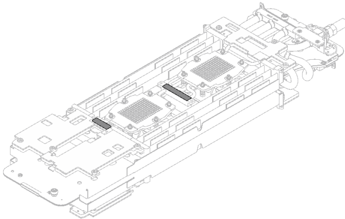
그림 26. 워터 루프 퍼티 패드
