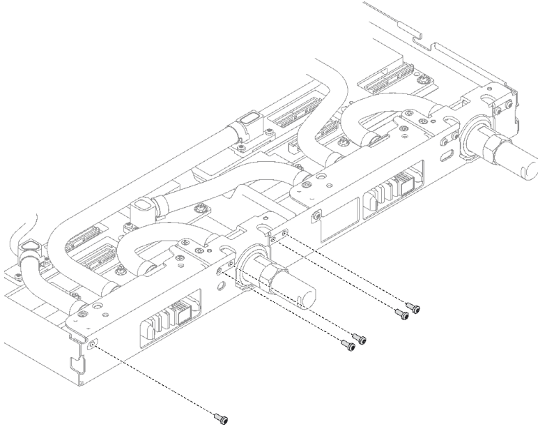
그림 194. 퀵 커넥트 나사 제거
