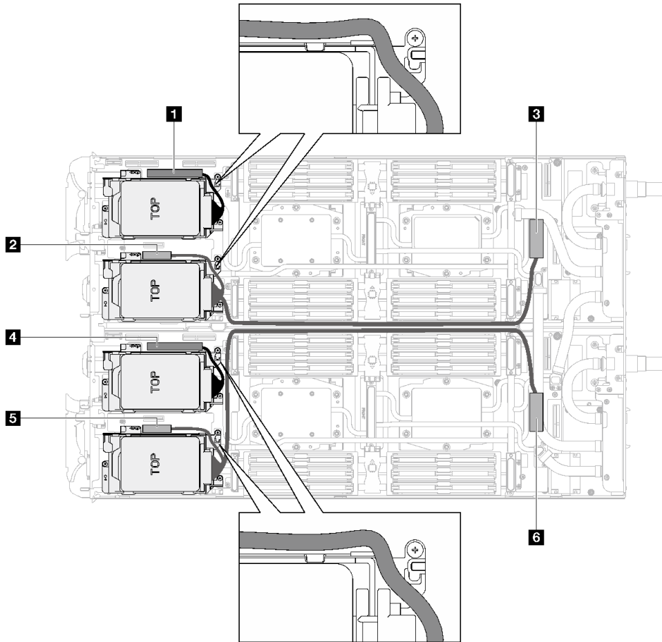
그림 79. SATA 드라이브용 드라이브 어셈블리 케이블 배선
