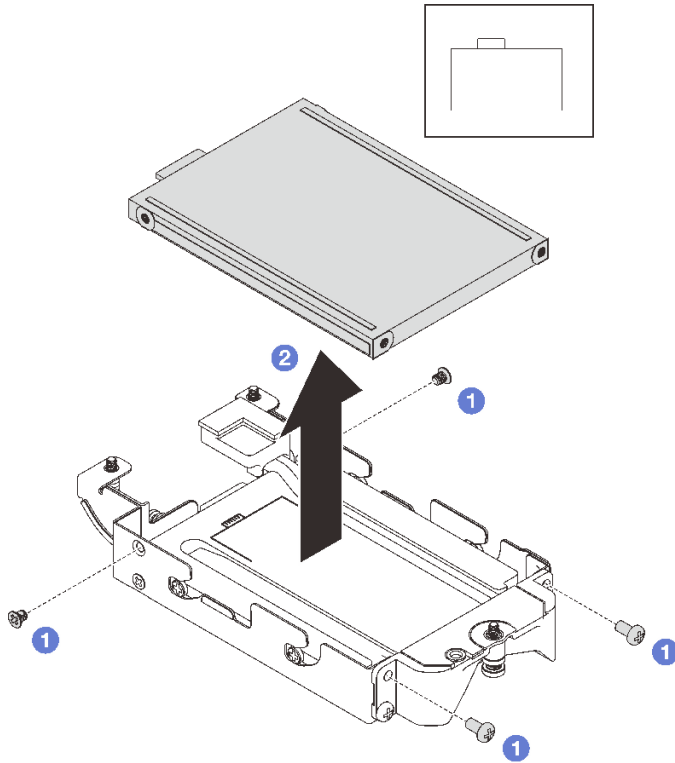
그림 102. 하단 E3.s 드라이브 제거
