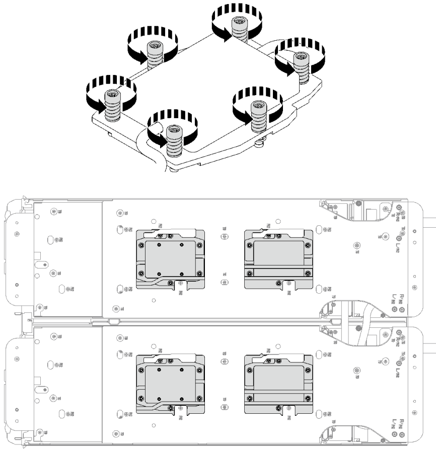
그림 224. 프로세서 냉각판 제거
