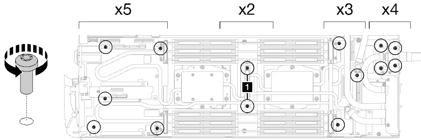
그림 220. 워터 루프 나사 제거
