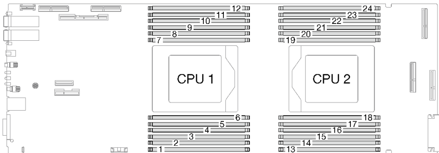
그림 1. 메모리 모듈 및 프로세서 레이아웃
