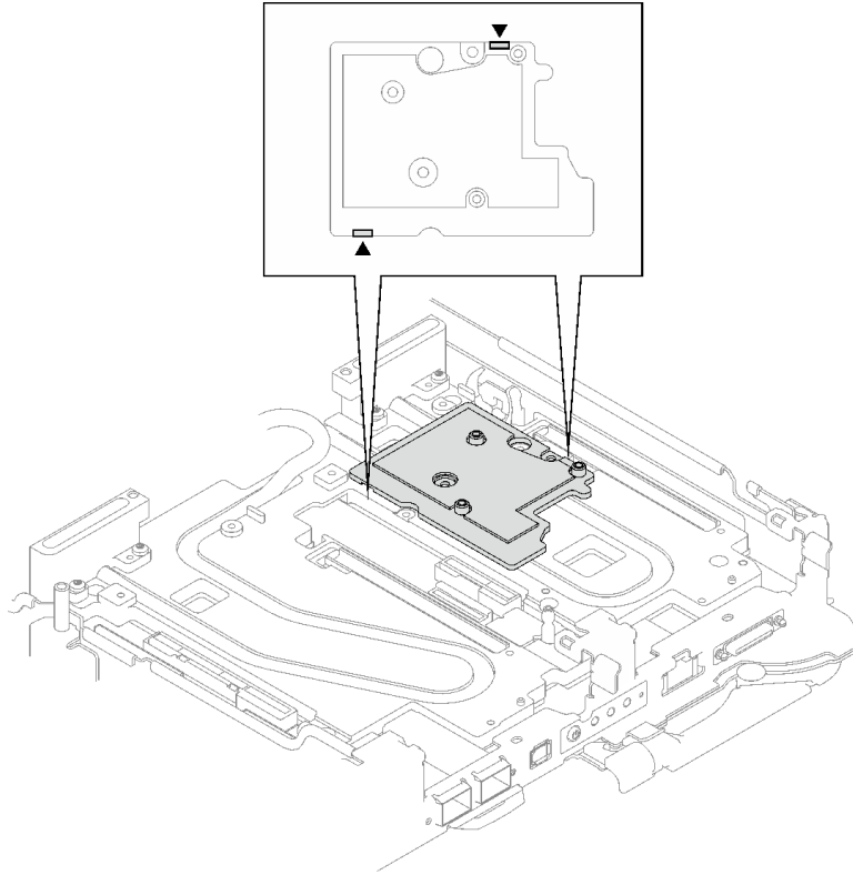
그림 183. 인터페이스판 하단의 구멍 위치
