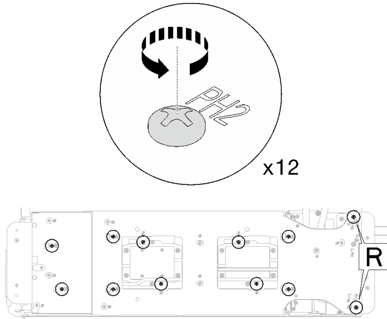
그림 238. 워터 루프 캐리어 나사 풀기
