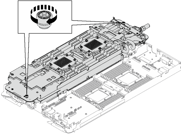
그림 19. 고정 나비 나사 조이기
