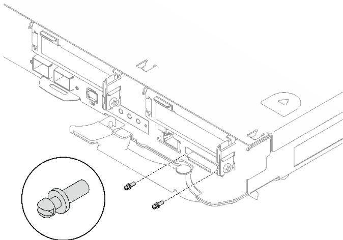
그림 277. KVM 나사 설치
