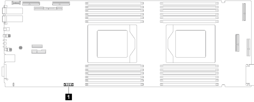
그림 46. CMOS 배터리 위치
