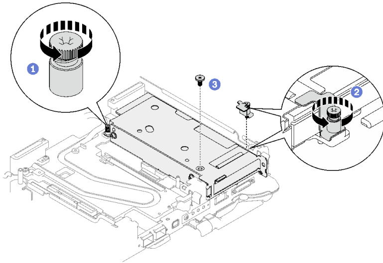
그림 150. 클램프 브래킷 고정 나사 제거
