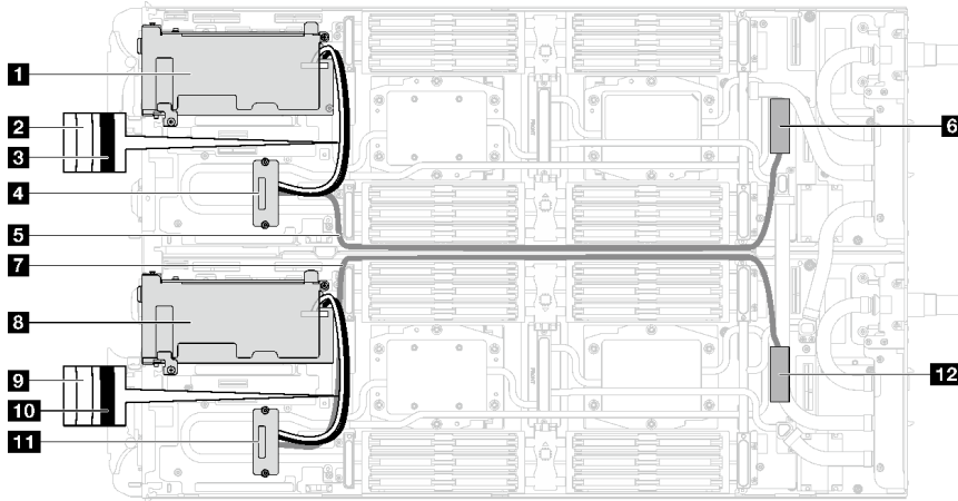
그림 284. 소켓 다이렉트 구성 케이블 배선
