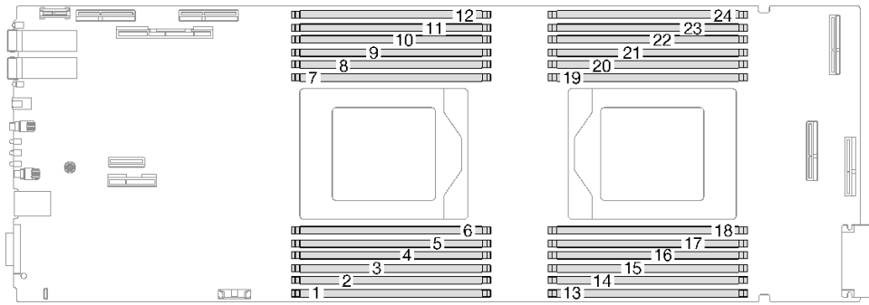
그림 129. 메모리 모듈 커넥터 위치
