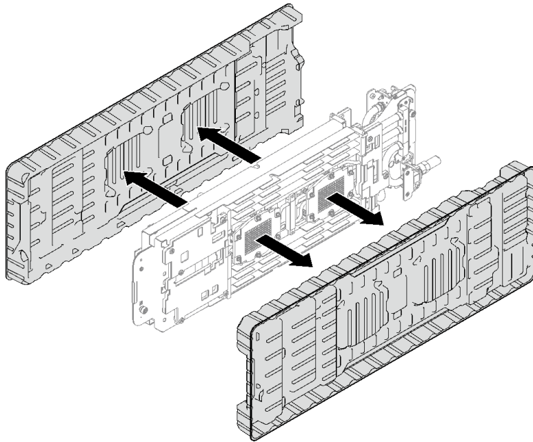
그림 22. 플라스틱 그리스 덮개 제거
