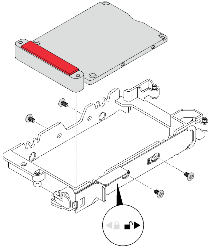
그림 68. 전도판 설치
