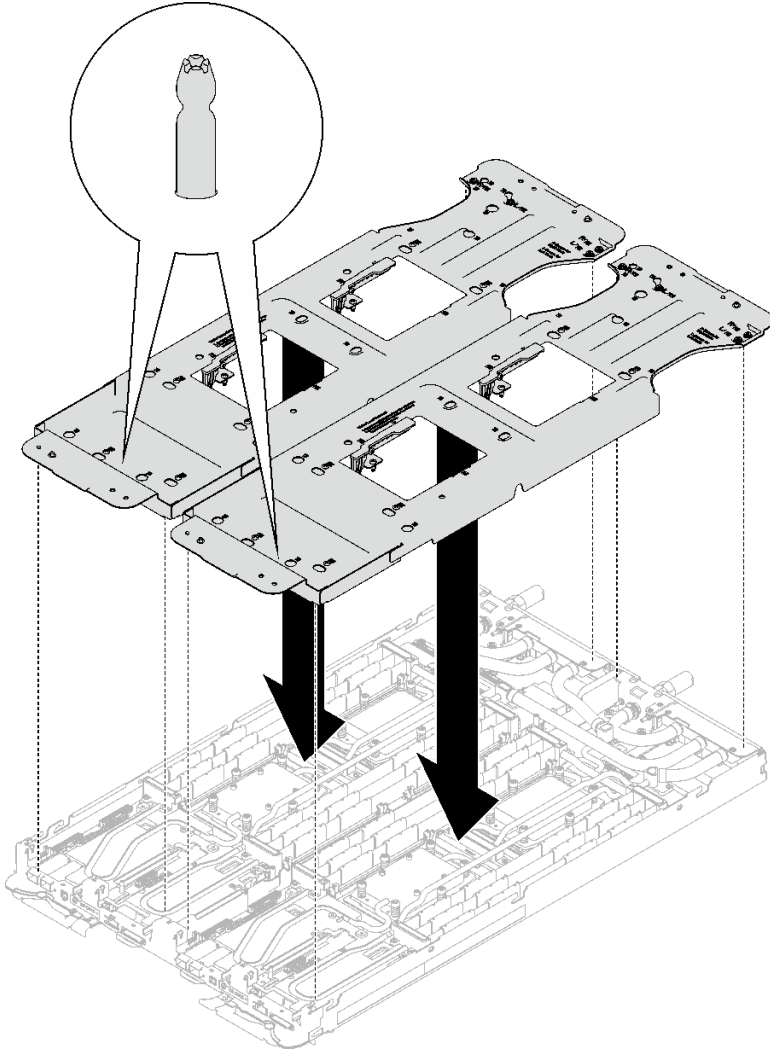
그림 13. 워터 루프 캐리어 설치
