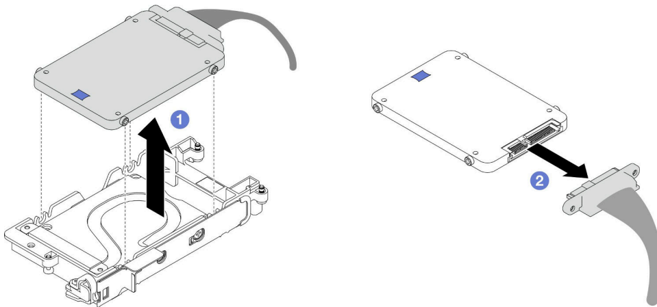
그림 85. 하단 드라이브 제거
