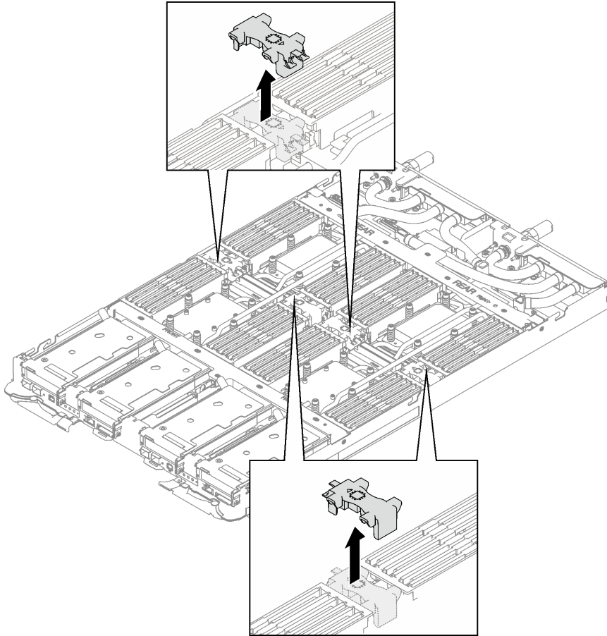
그림 51. DIMM 콤 제거
