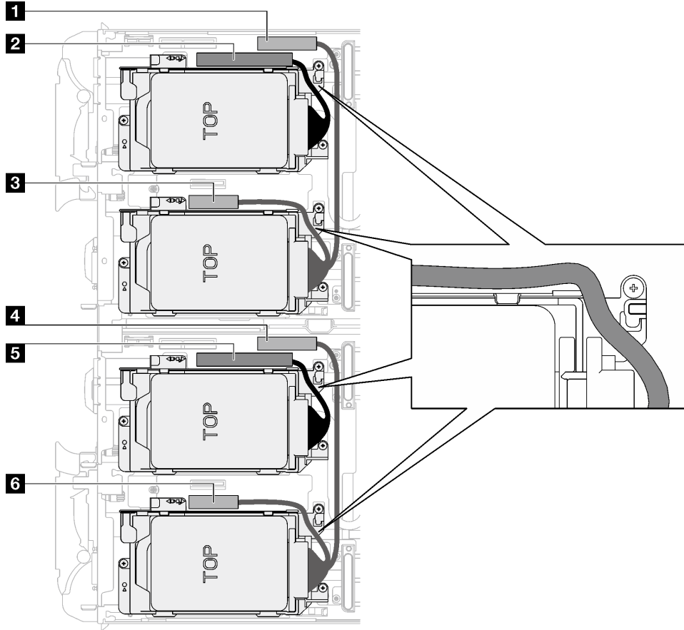
그림 95. 모든 NVMe 드라이브용 드라이브 어셈블리 케이블 배선
