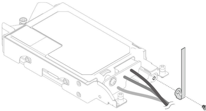
그림 100. 케이블 타이 제거
