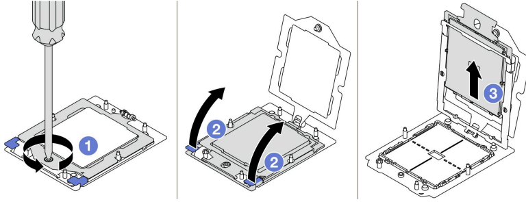
그림 227. 프로세서 제거
