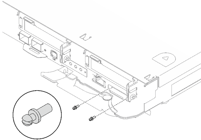
그림 267. KVM 나사 설치
