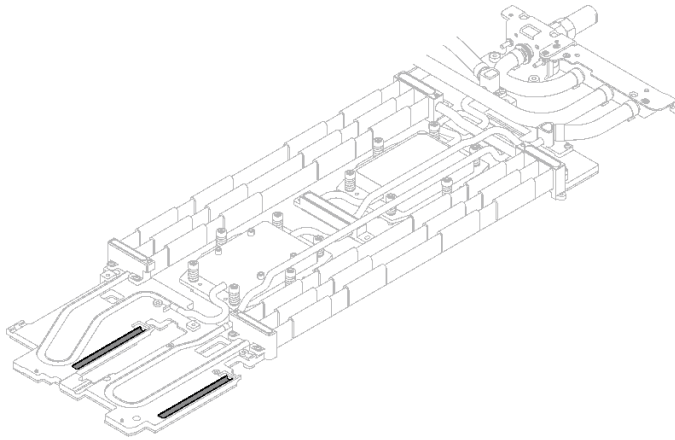
그림 233. 워터 루프 갭 패드(상단)
