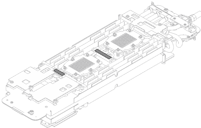
그림 234. 워터 루프 퍼티 패드
