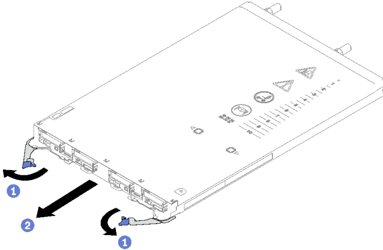
그림 4. 트레이 제거
