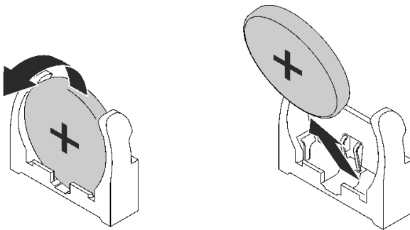
그림 47. CMOS 배터리 제거
