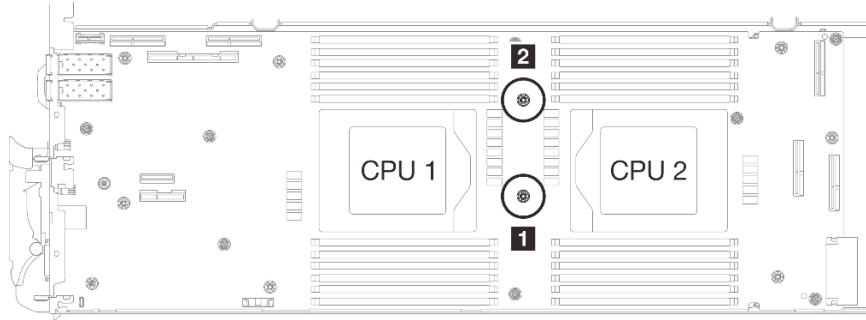
그림 251. 차폐 케이블 1/2 및 3의 나사 구멍 위치
