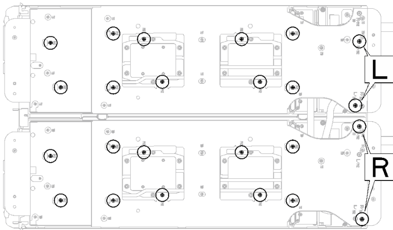
그림 31. 워터 루프 캐리어 나사 풀기
