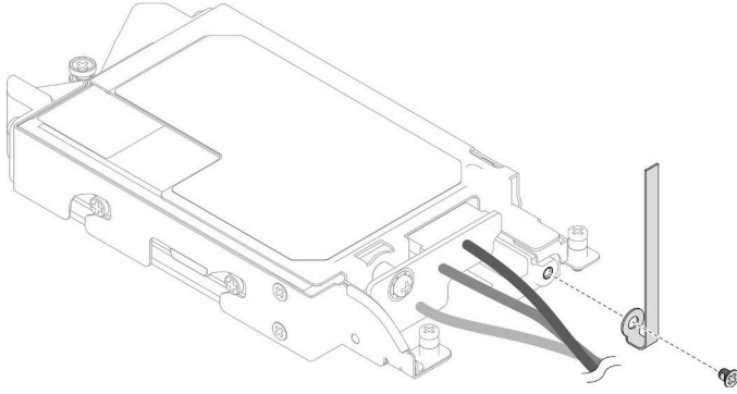
그림 111. 케이블 타이 설치
