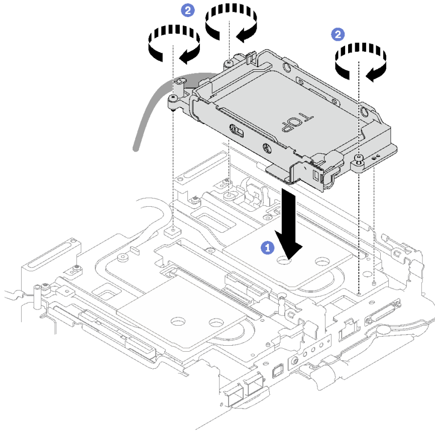
그림 76. 7mm 드라이브 케이지 어셈블리 1개 설치
