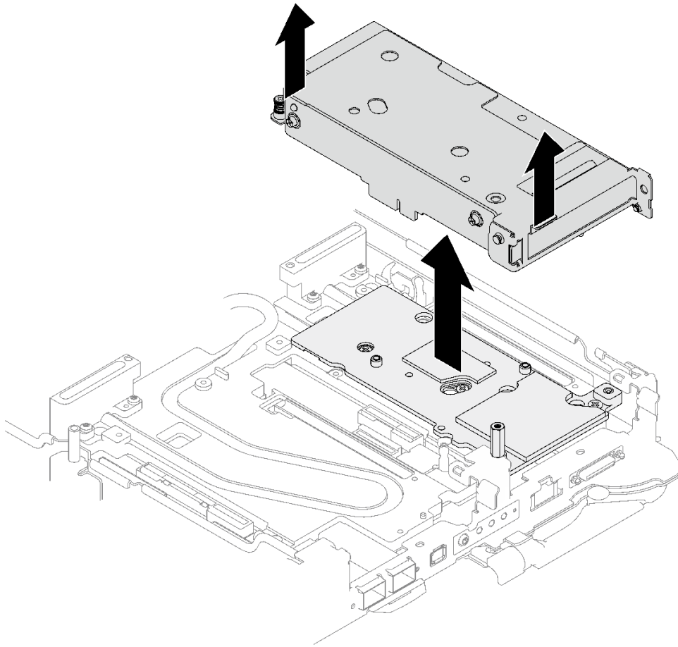
그림 164. PCIe 라이저 어셈블리 제거
