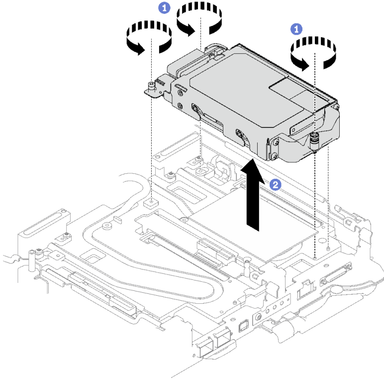
그림 97. E3.s 드라이브 케이지 어셈블리 제거
