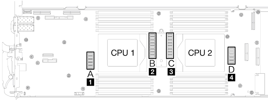
그림 261. 시스템 보드의 인덕터 위치
