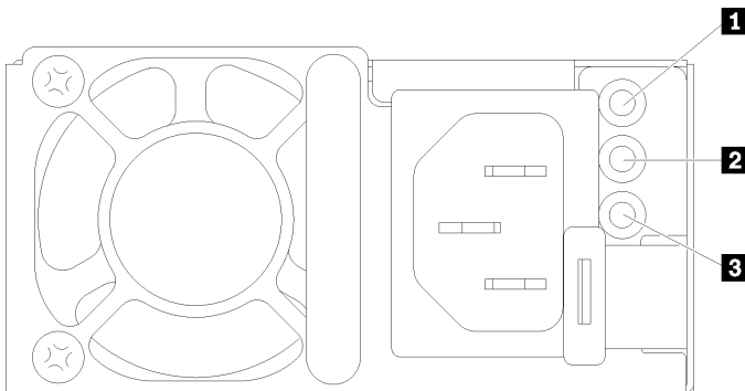
그림 290. AC 전원 공급 장치 LED
