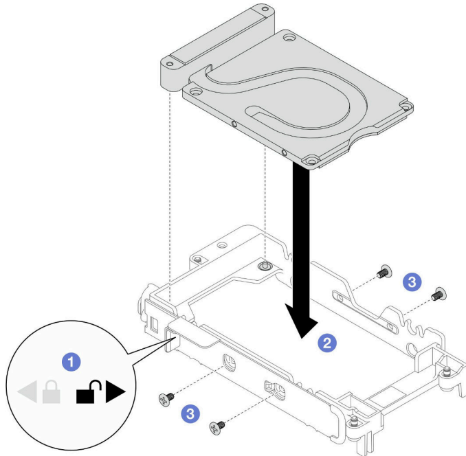
그림 87. 전도판 설치
