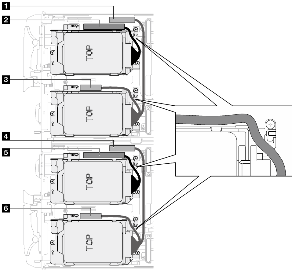
그림 55. 모든 NVMe 드라이브용 드라이브 어셈블리 케이블 배선
