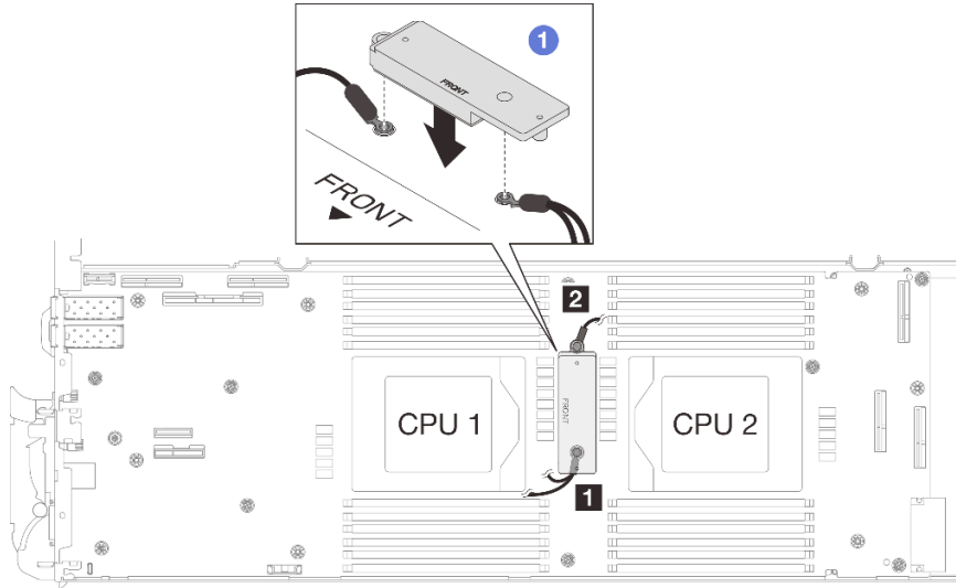
그림 270. VR 전도판, 차폐 케이블 및 시스템 보드 나사 구멍 맞추기
