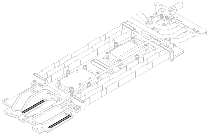
그림 207. 워터 루프 캡 패드(상단)
