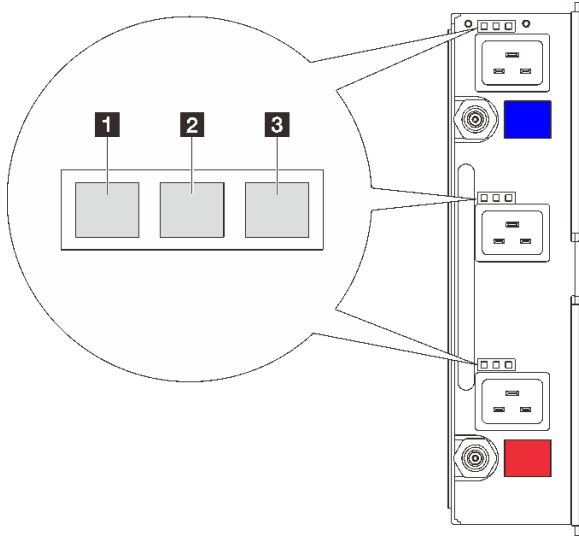
그림 291. DWC 전원 공급 장치 LED
