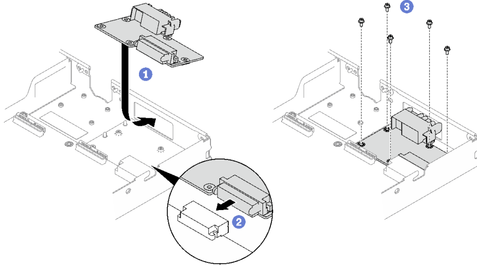
그림 204. 전원 분배 보드 설치
