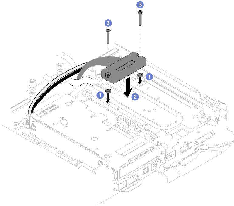
그림 193. 상호 연결 케이블 설치
