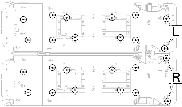
그림 14. 워터 루프 캐리어 나사 설치
