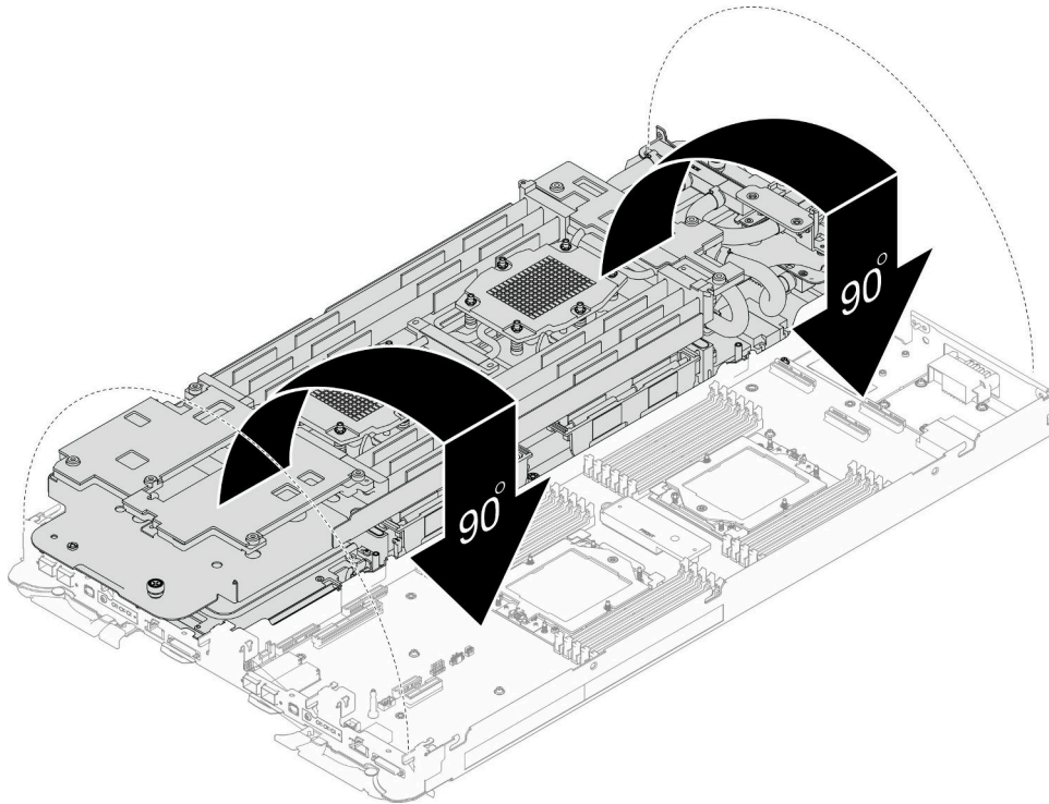
그림 236. 워터 루프 설치
