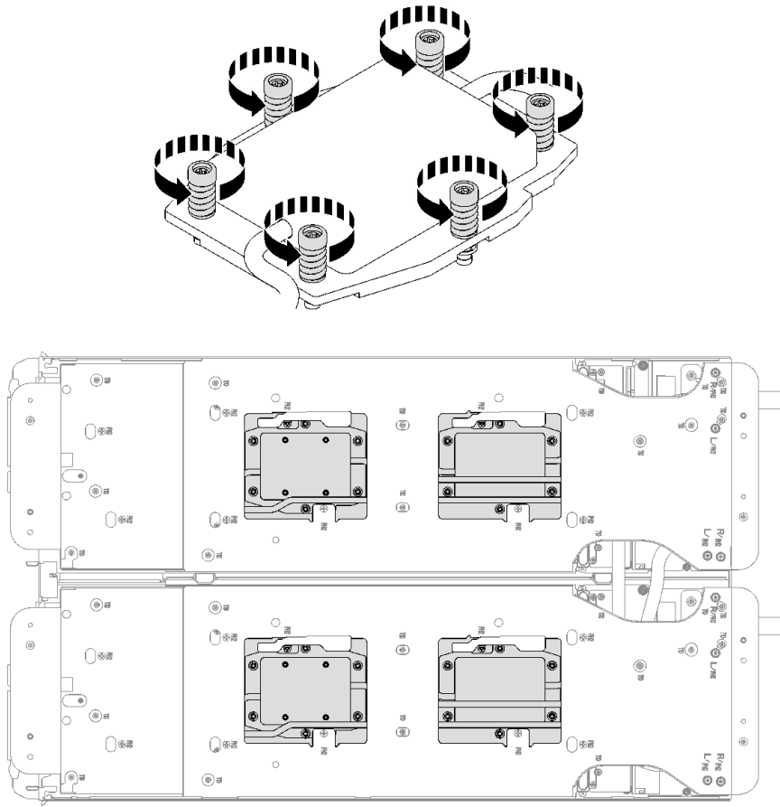
그림 200. 프로세서 냉각판 제거
