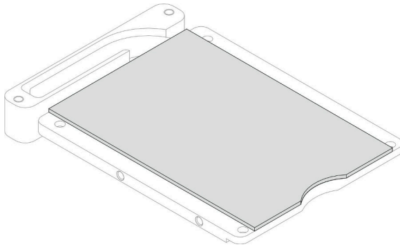
그림 86. 전도판 갭 패드 설치
