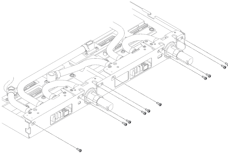
그림 10. 퀵 커넥트 나사 제거
