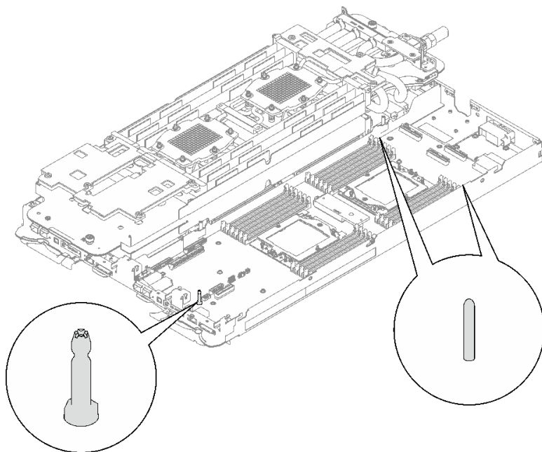
그림 235. 오른쪽 컴퓨팅 노드의 가이드 핀
