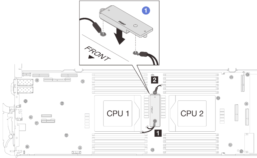
그림 253. VR 전도판, 차폐 케이블 및 시스템 보드 나사 구멍 맞추기
