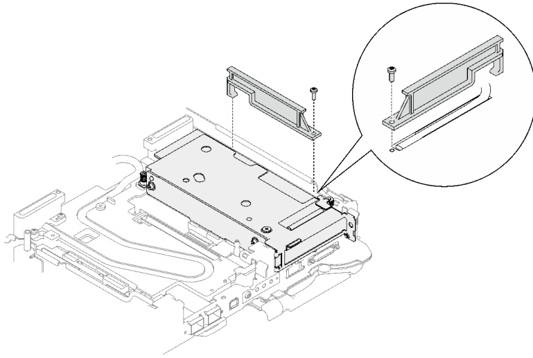
그림 149. 히트파이프 빔 제거
