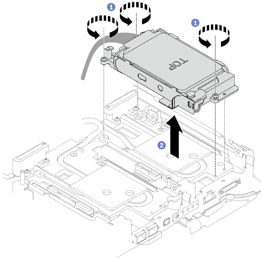
그림 57. 7mm 드라이브 케이지 어셈블리 2개 제거
