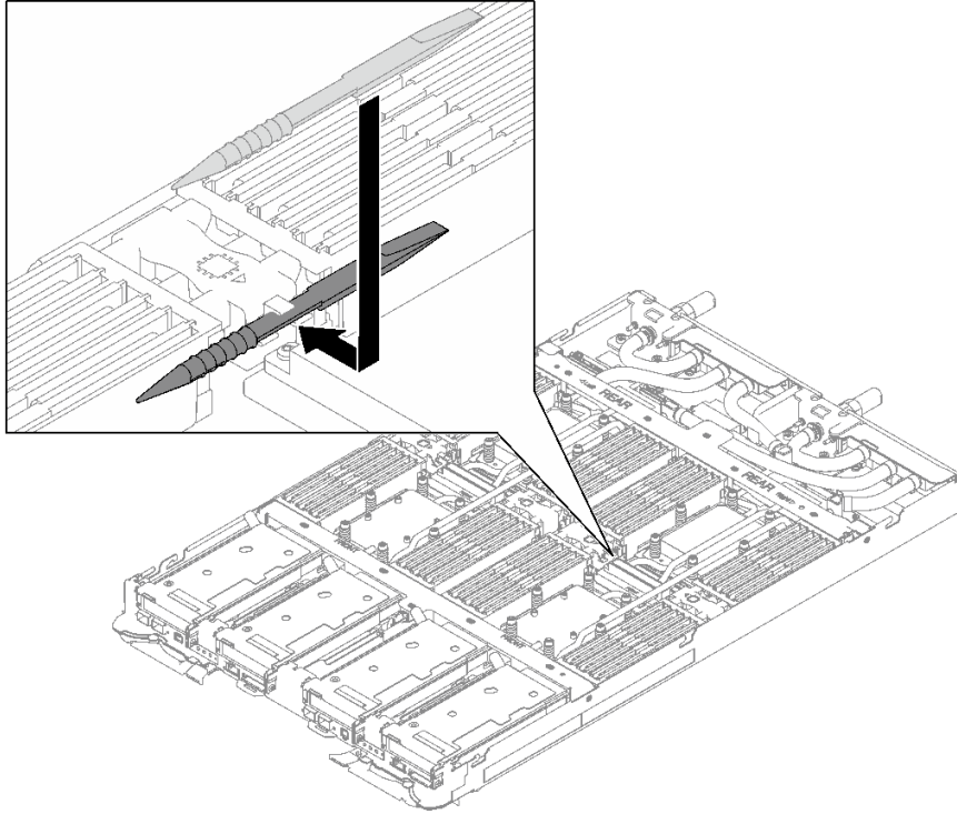
그림 142. 메모리 모듈 도구 설치
