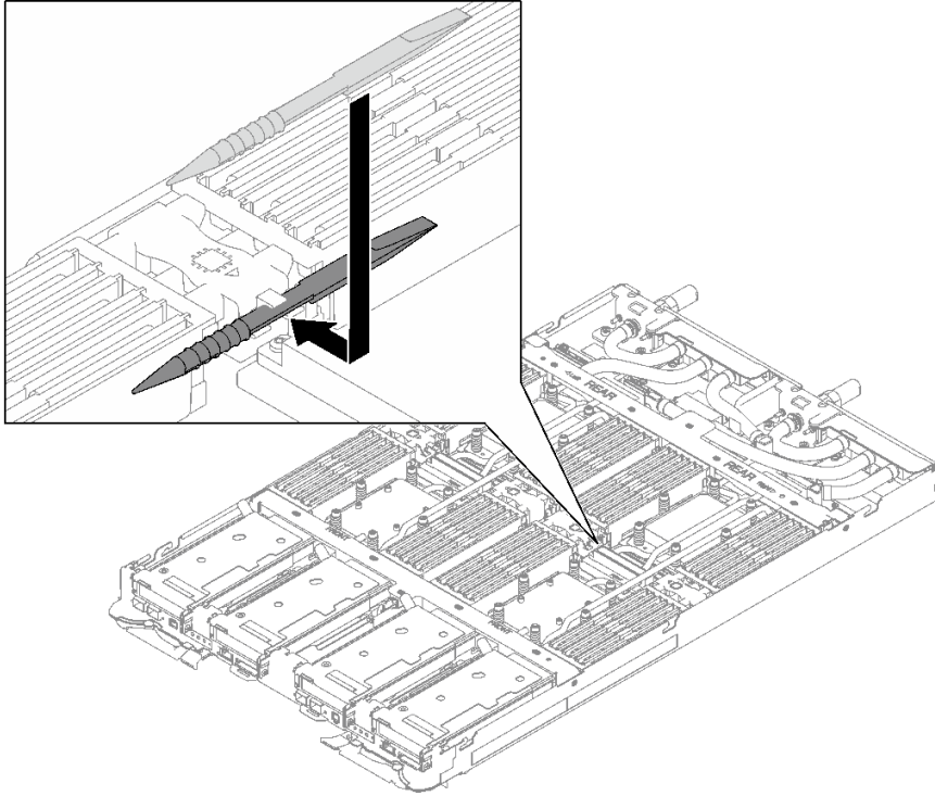
그림 135. 메모리 모듈 도구 설치
