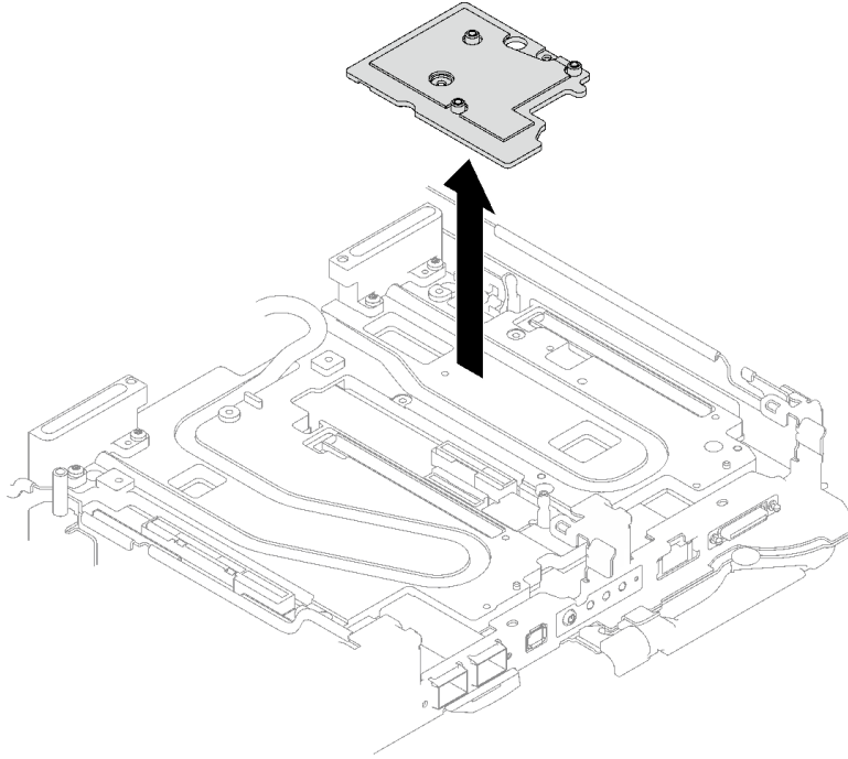
그림 185. 인터페이스판 제거
