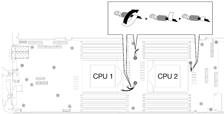
그림 258. 차폐 케이블에 레이블 감기
