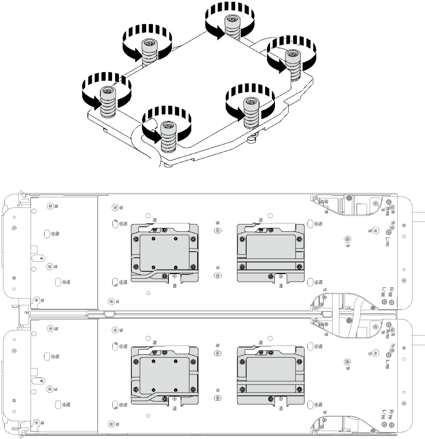
그림 16. 프로세서 냉각판 제거
