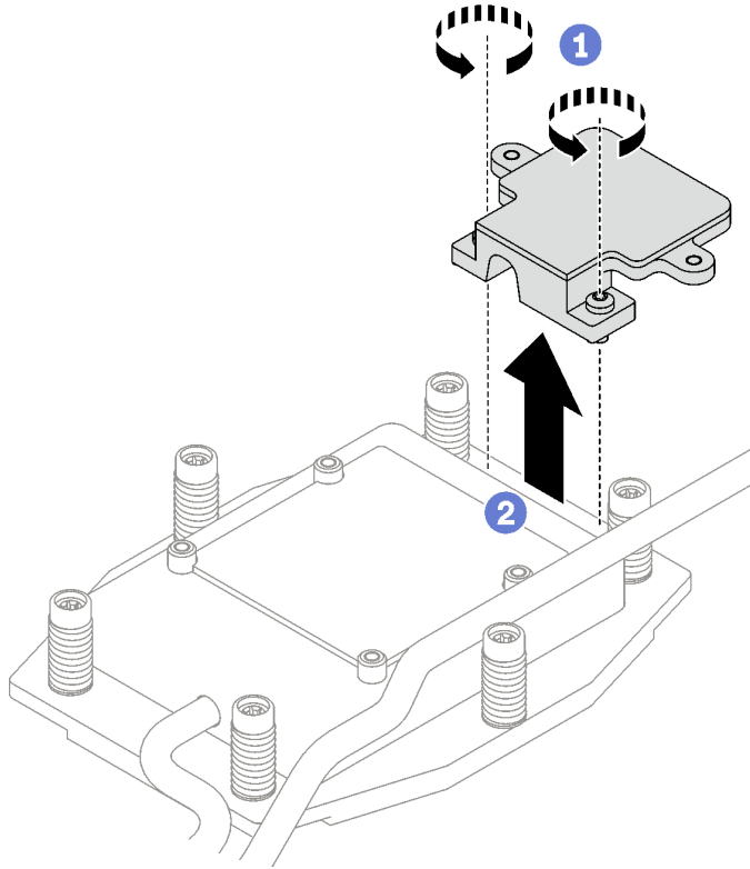
그림 120. M.2 백플레인 냉각판 제거
