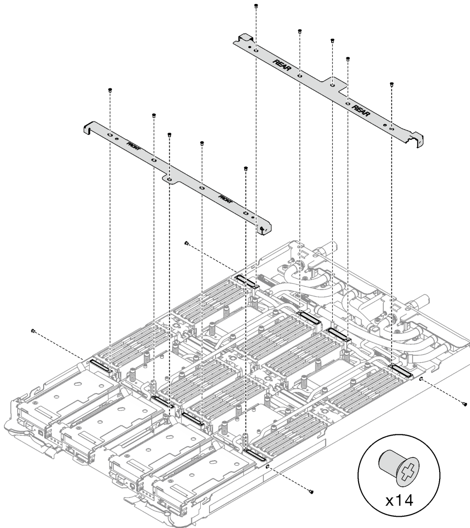
그림 8. 십자형 브레이스 제거
