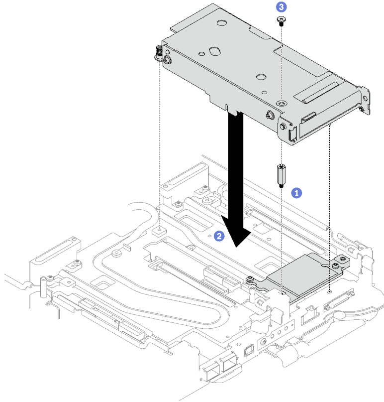
그림 159. PCIe 라이저 어셈블리 설치
