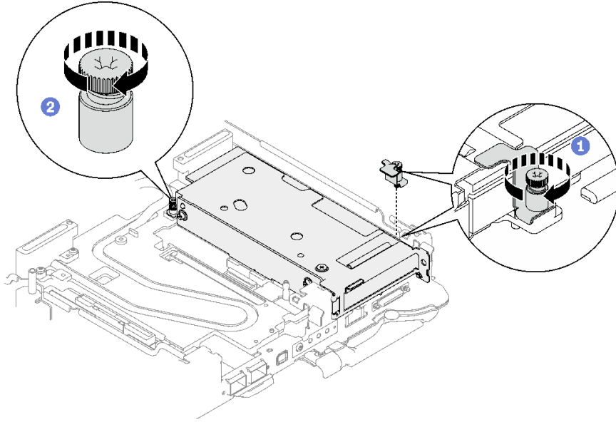
그림 160. 클램프 브래킷 고정 나사 설치
