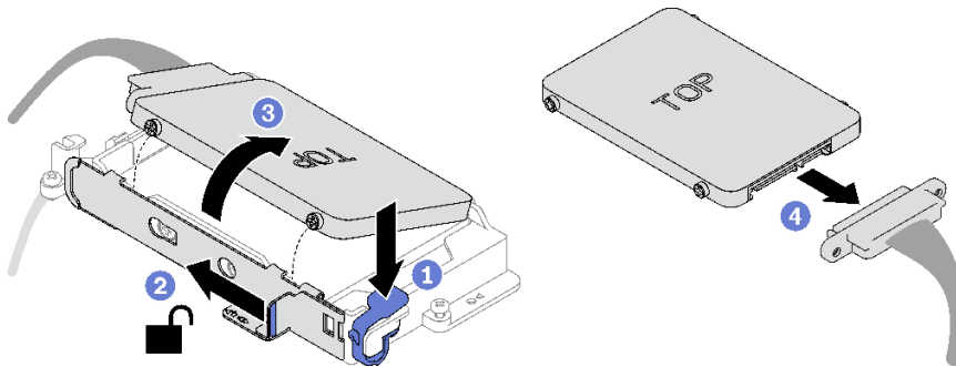
그림 62. 상단 드라이브 제거
