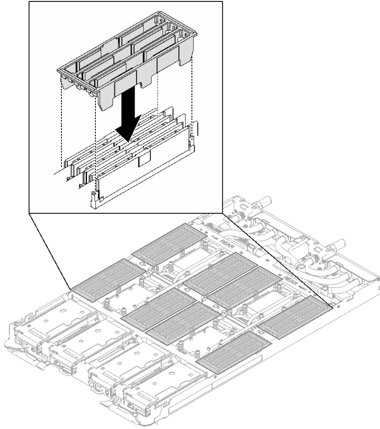
그림 141. DIMM 덮개 설치
