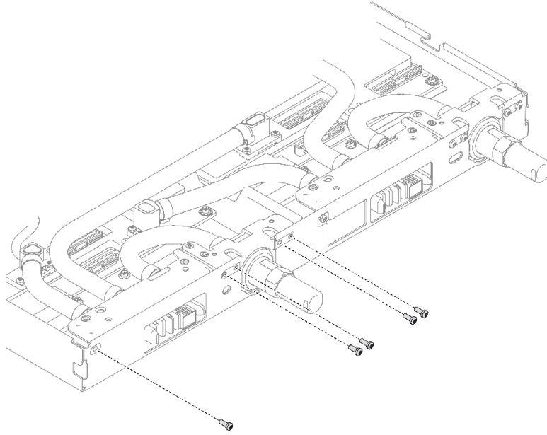
그림 242. 클릭 커넥트 나사 설치
