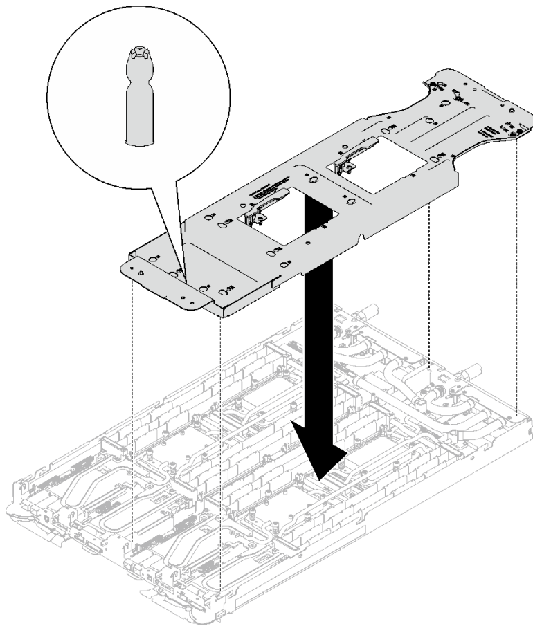
그림 197. 워터 루프 캐리어 설치
