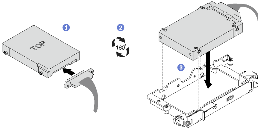
그림 66. 15mm 드라이브 설치
