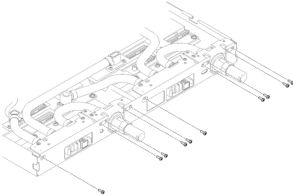
그림 35. 퀵 커넥트 나사 설치
