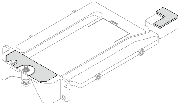
그림 107. 전도판 퍼티 패드 교체
