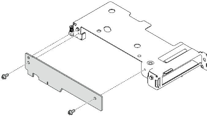
그림 170. 확장 보드 제거
