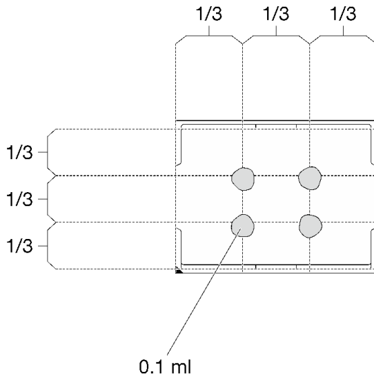
그림 230. 열전도 그리스 도포
