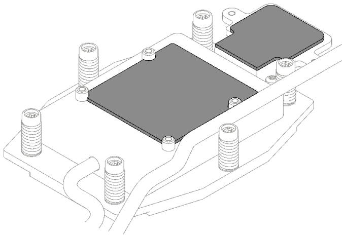
그림 126. 프로세서 냉각판 및 M.2 냉각판의 퍼티 패드
