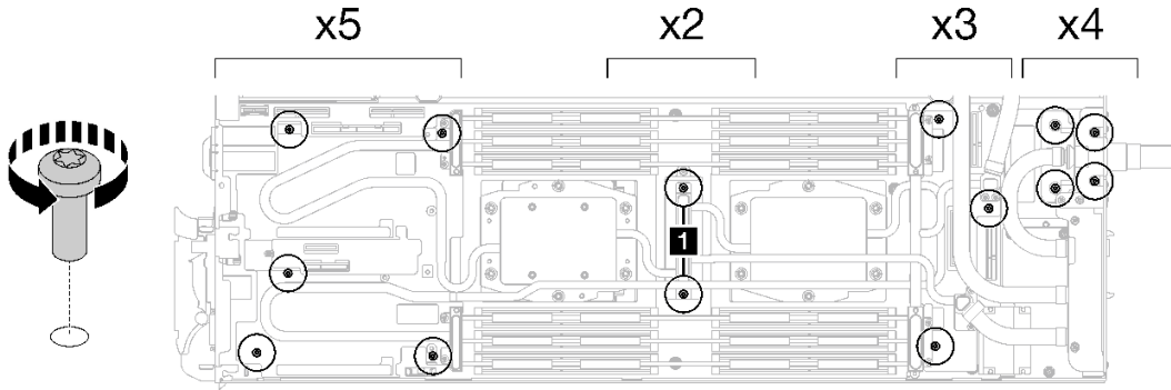
그림 12. 워터 루프 나사 제거
