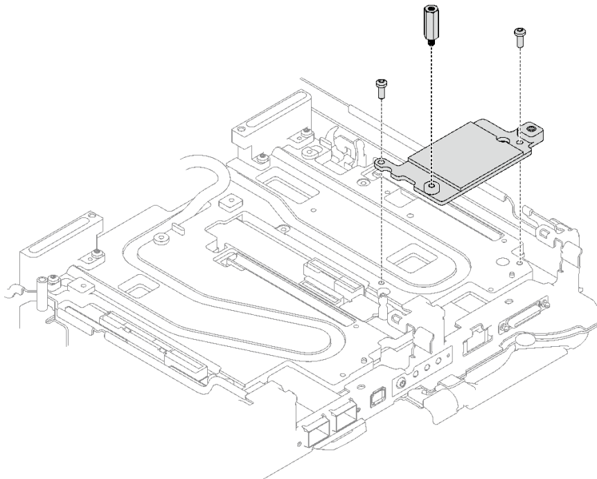
그림 152. 인터페이스판 제거
