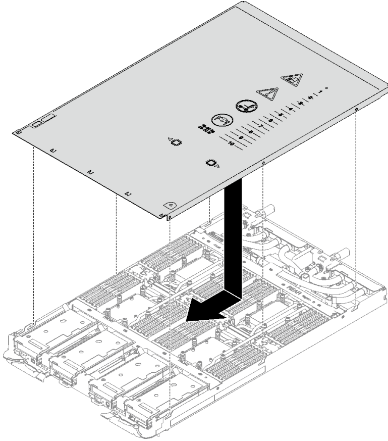
그림 7. 트레이 덮개 설치
