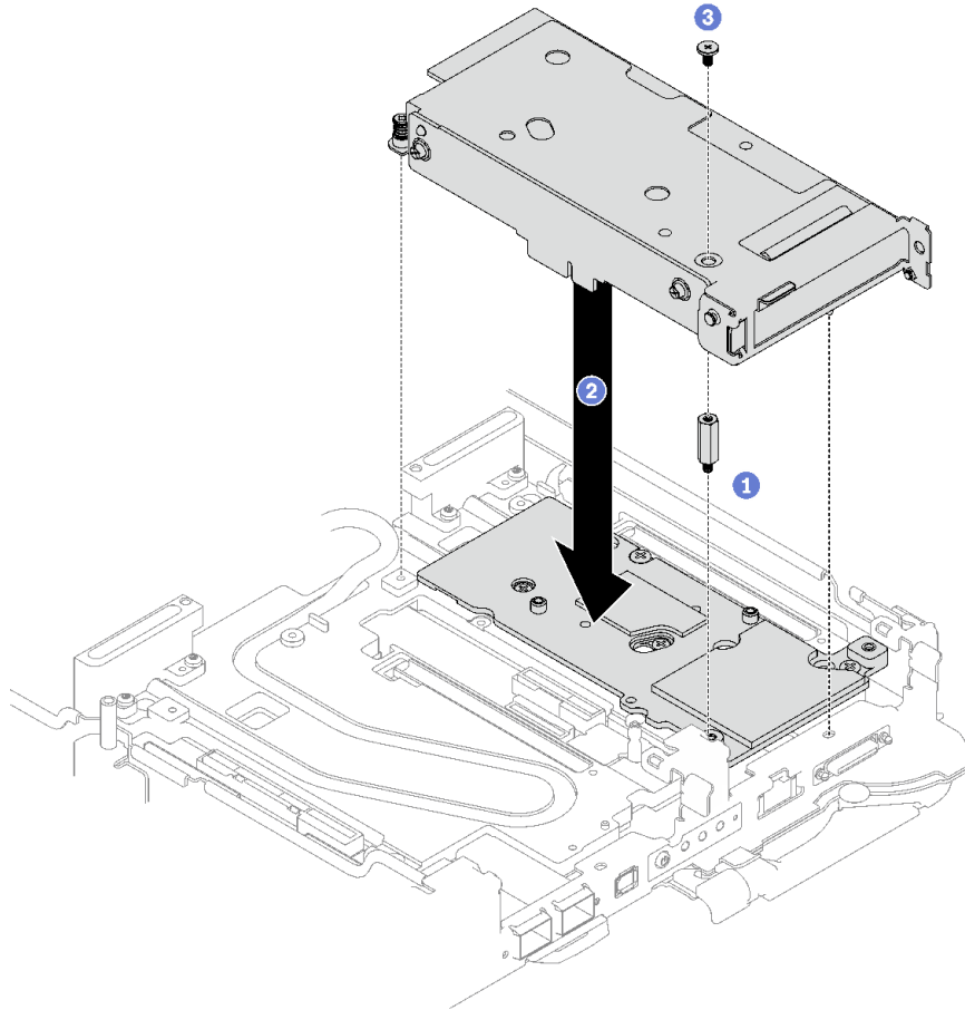
그림 175. PCIe 라이저 어셈블리 설치
