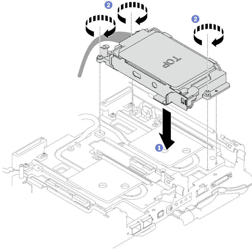
그림 77. 7mm 드라이브 케이지 어셈블리 2개 설치
