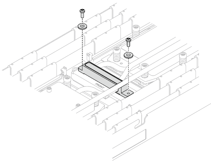
그림 195. 와셔가 있는 VR 냉각판 나사
