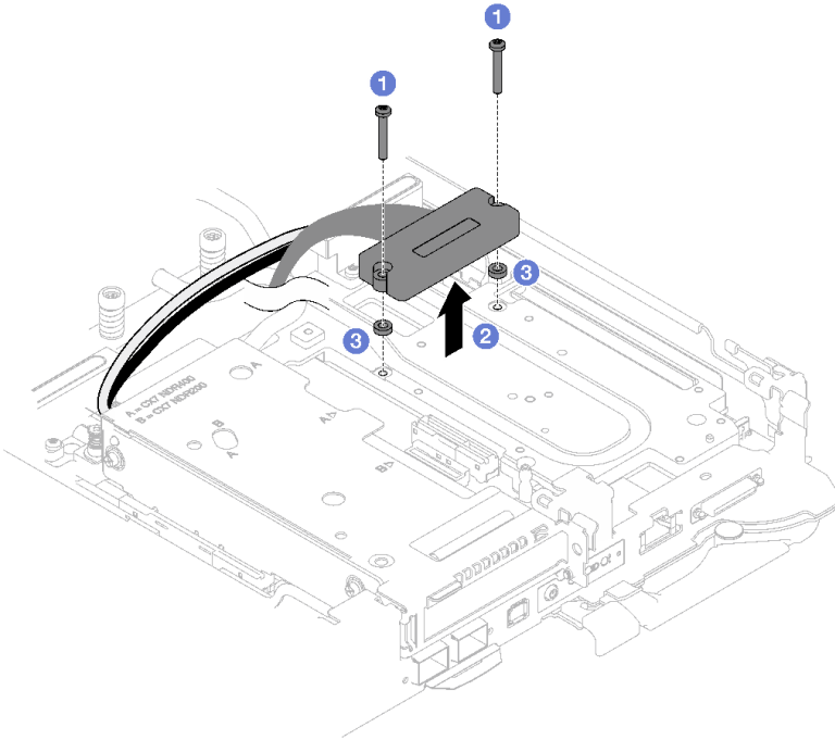
그림 162. 상호 연결 케이블 제거
