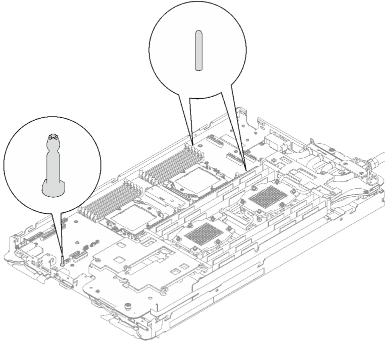
그림 28. 왼쪽 컴퓨팅 노드의 가이드 핀
