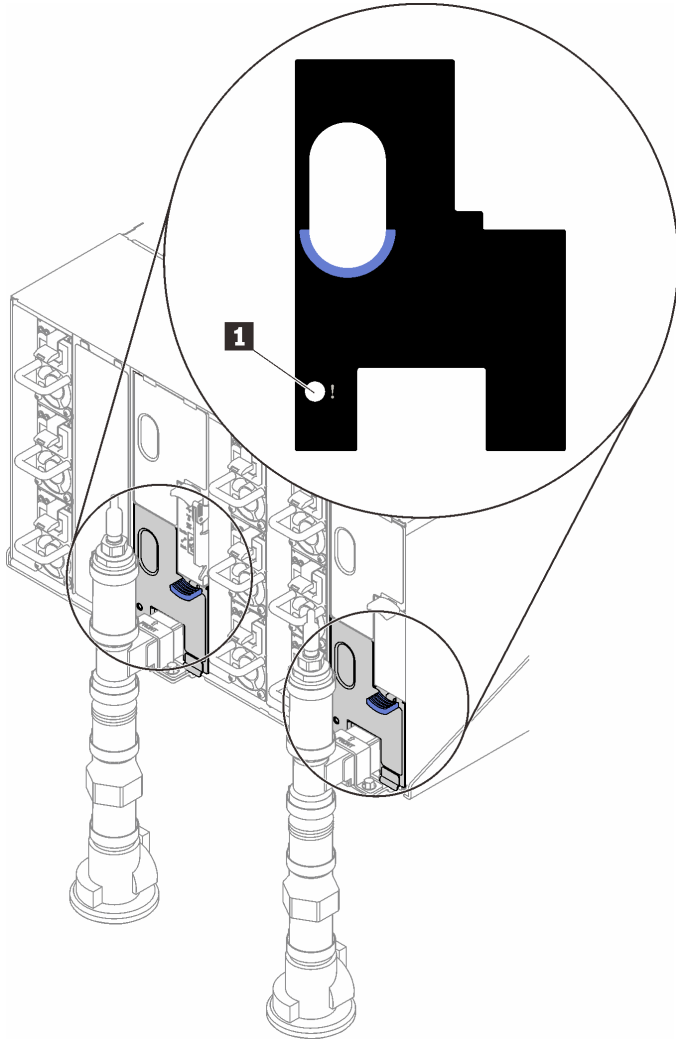
그림 294. 드립 센서 LED
