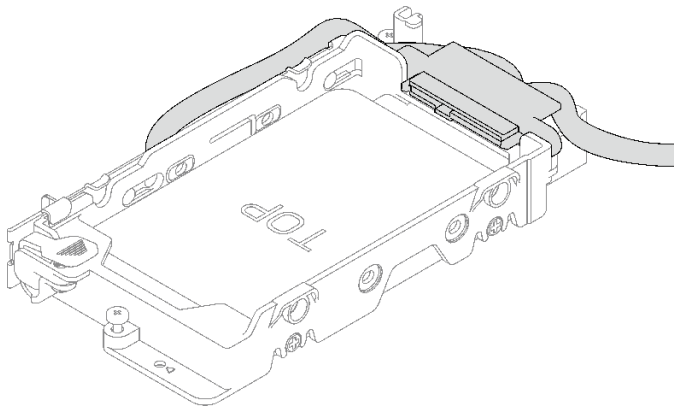
그림 67. 분리된 케이블 플러저 고정
