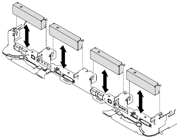
그림 83. 빈 베젤 필터 제거
