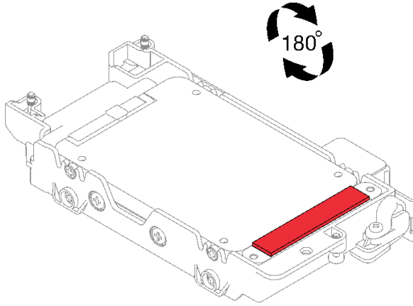
그림 72. 겹 패드 위치
