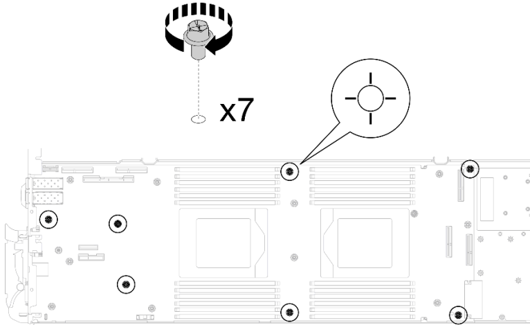
그림 276. 시스템 보드 나사 설치
