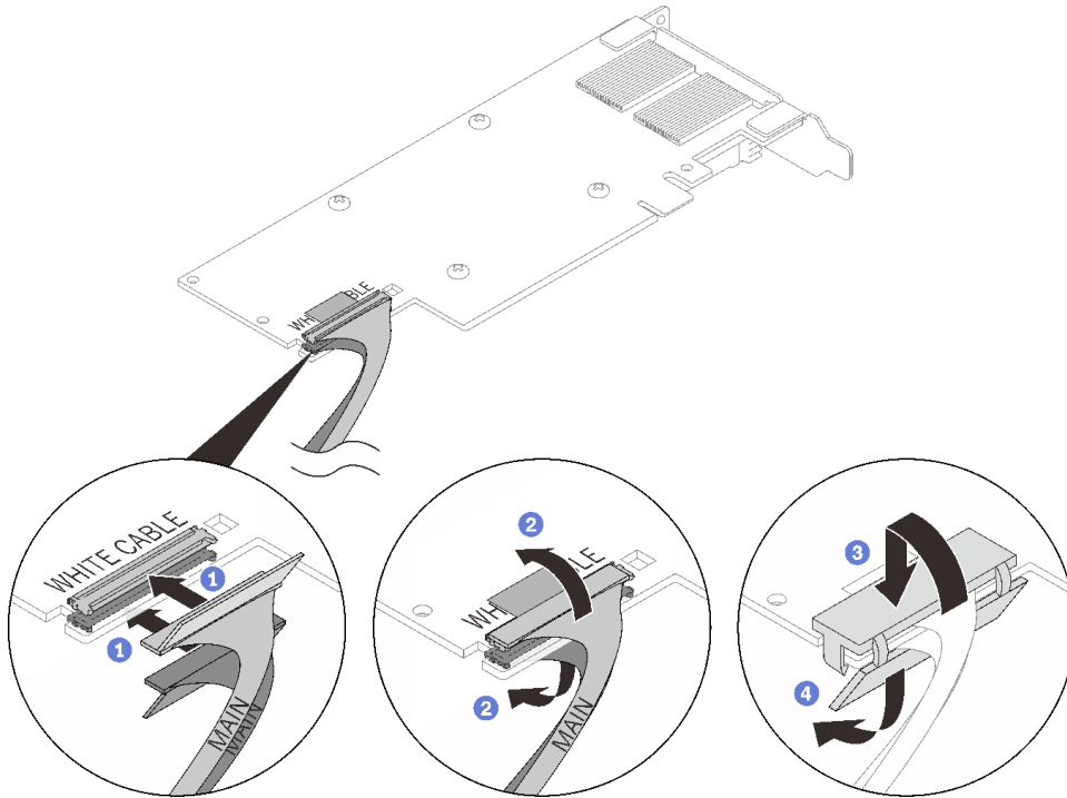
그림 147. PCIe 어댑터 케이블 설치
