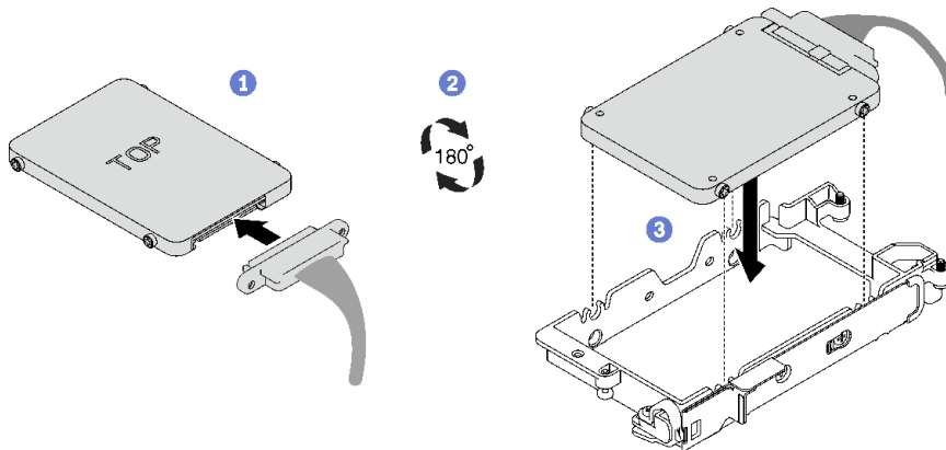
그림 65. 7mm 드라이브 설치
