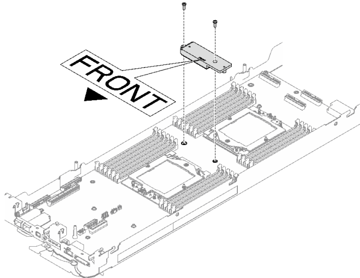
그림 43. VR 전도판 제거
