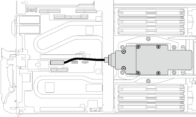
그림 118. M.2 백플레인 어셈블리 케이블 제거
