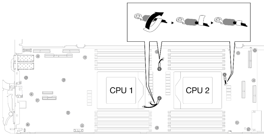
그림 275. 차폐 케이블에 레이블 감기
