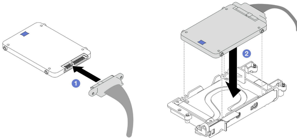
그림 88. 아래쪽 드라이브 설치
