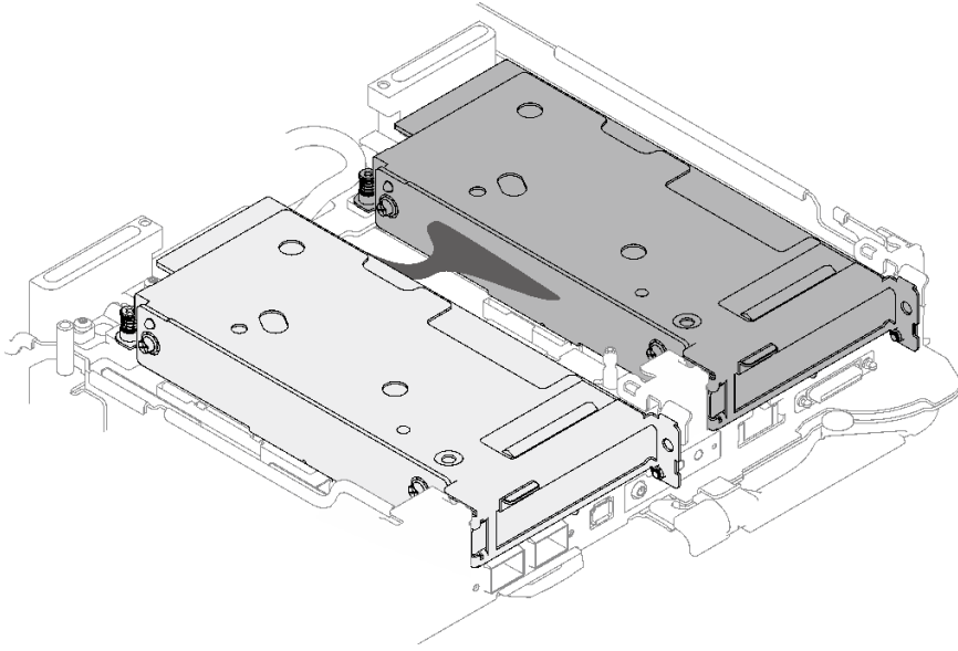
그림 188. 슬롯 1 및 슬롯 2에 설치되는 PCIe 라이저 유형
