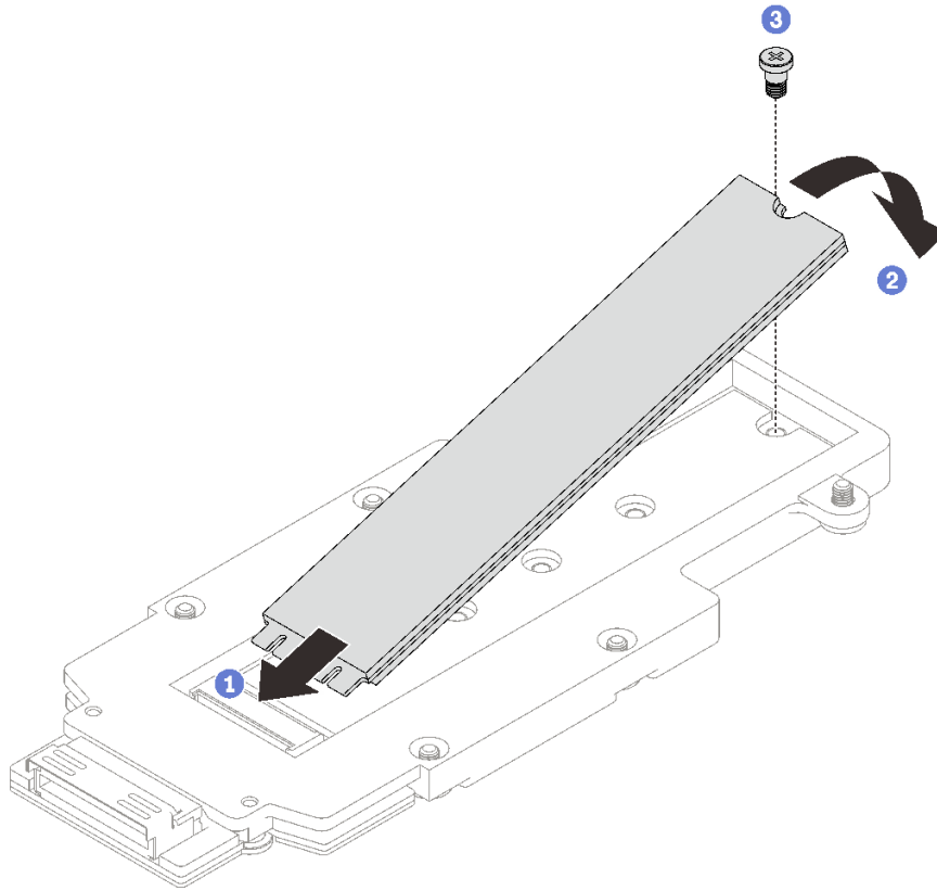
그림 123. M.2 드라이브 설치
