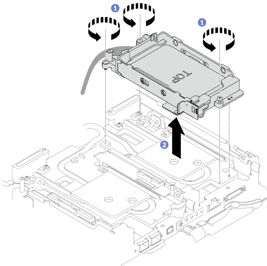
그림 56. 7mm 드라이브 케이징 어셈블리 1개 제거
