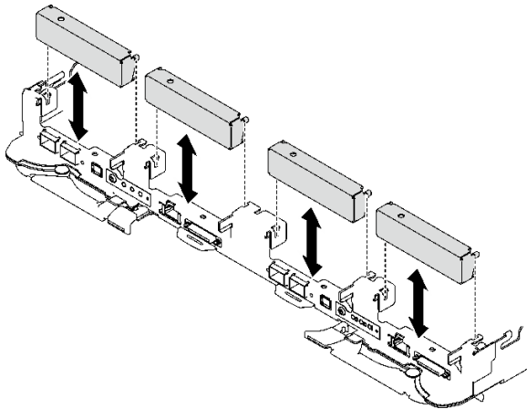
그림 71. 빈 베젤 필터 설치
