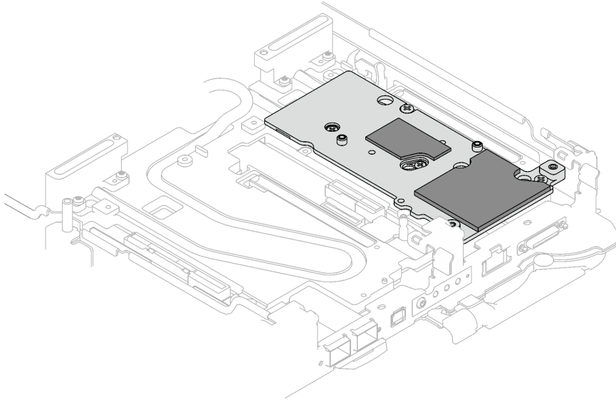
그림 174. CX-7 NDR 200용 냉각판의 인터페이스 패드
