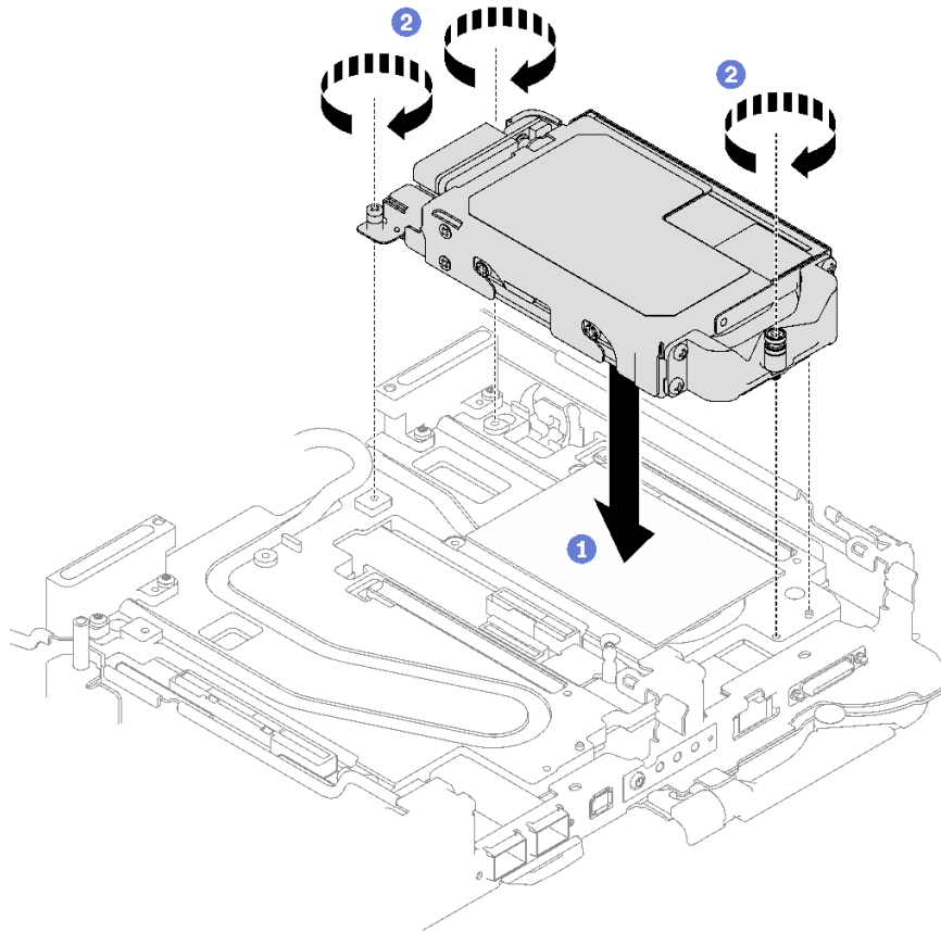
그림 116. E3.s 드라이브 케이지 어셈블리 설치
