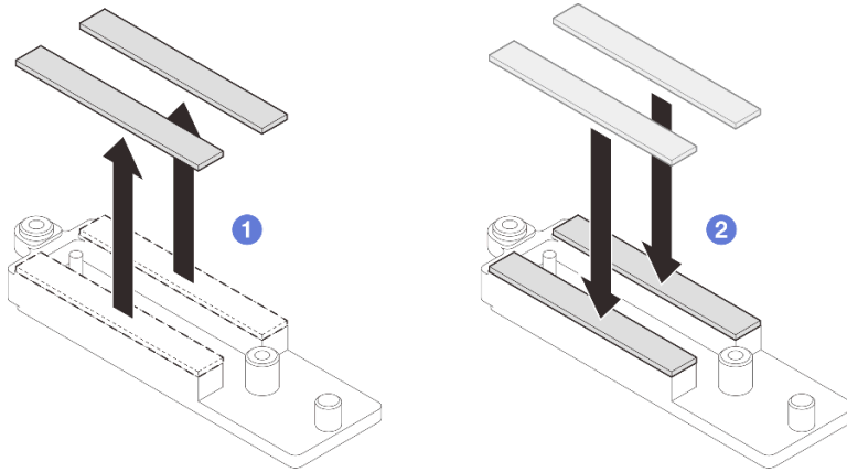
그림 278. VR 전도판 퍼티 패드 교체
