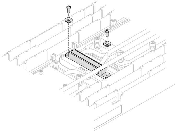
그림 214. 와셔가 있는 VR 냉각판 나사
