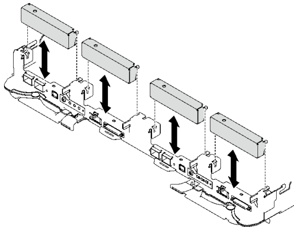
그림 59. 빈 베젤 필러 제거
