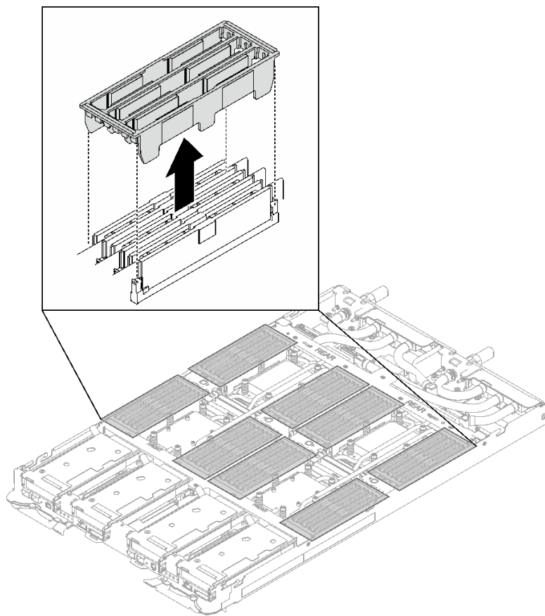
그림 138. DIMM 덮개 제거
