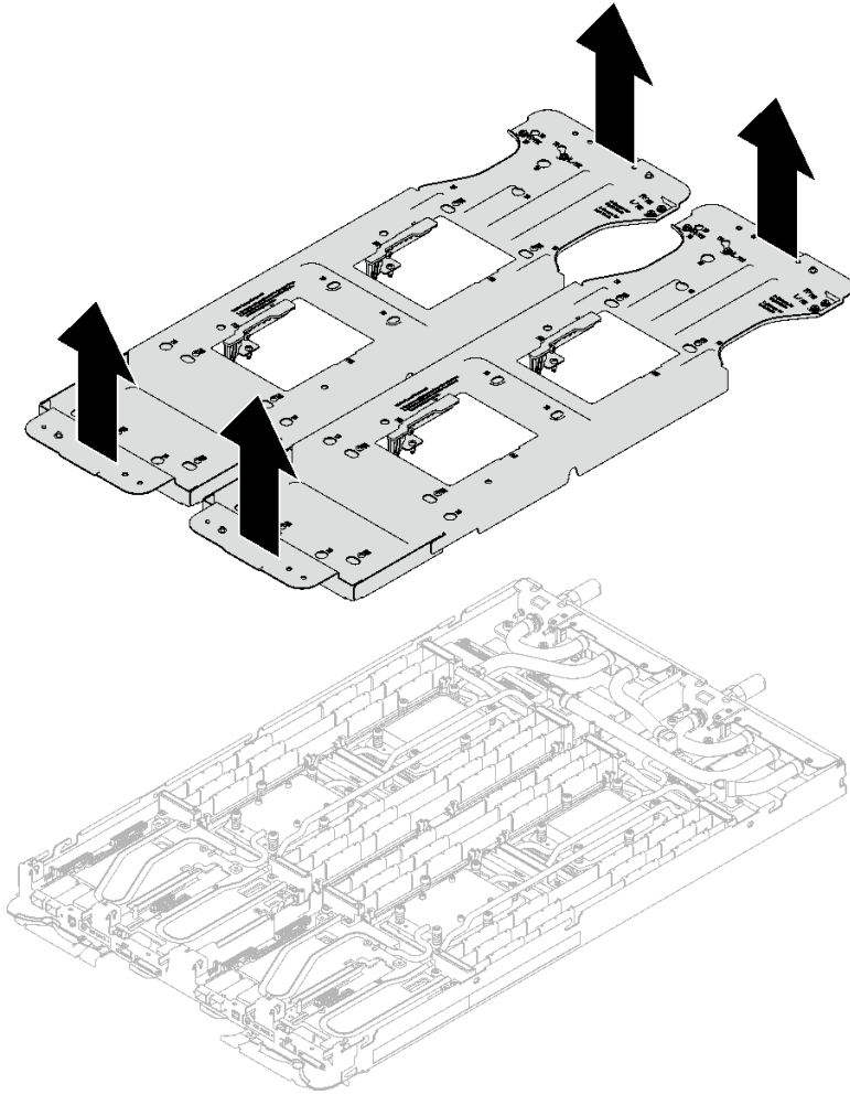
그림 32. 워터 루프 캐리어 제거
