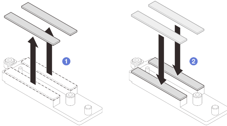
그림 248. VR 전도판 퍼티 패드 교체
