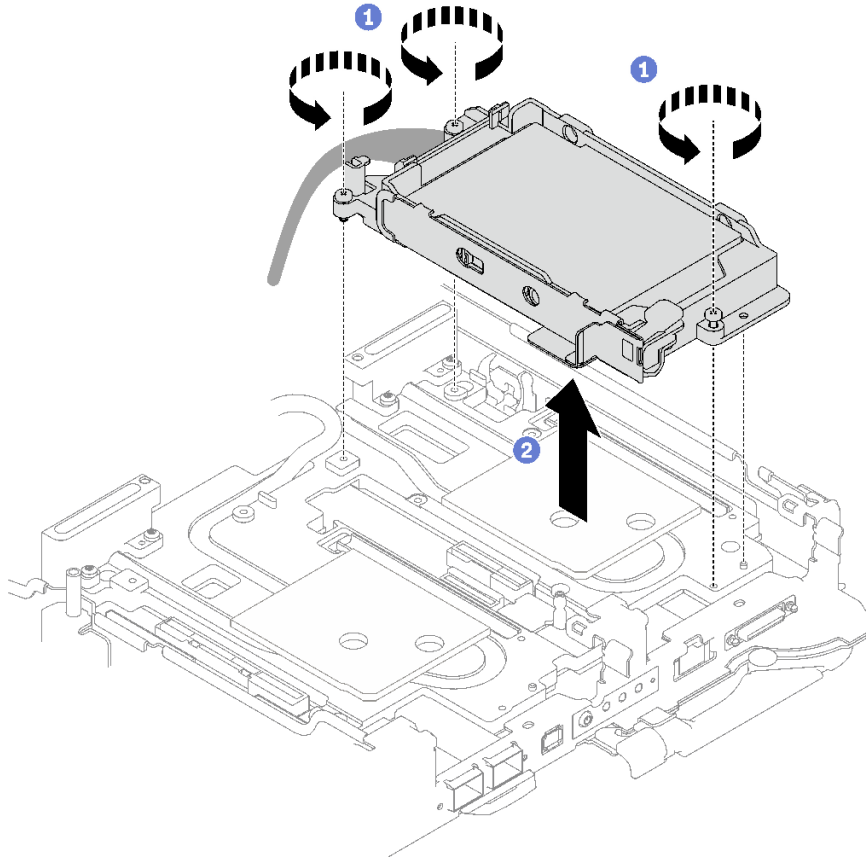
그림 58. 15mm 드라이브 케이지 어셈블리 1개 제거
