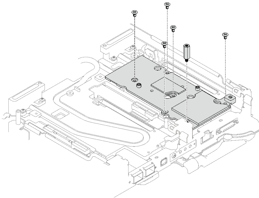
그림 173. 인터페이스판 설치
