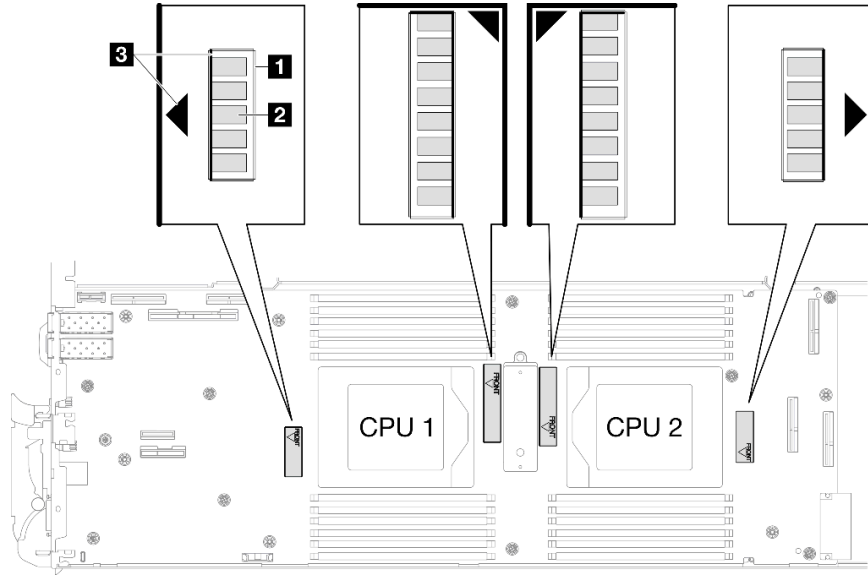
그림 263. 인덕터 부착 지점
