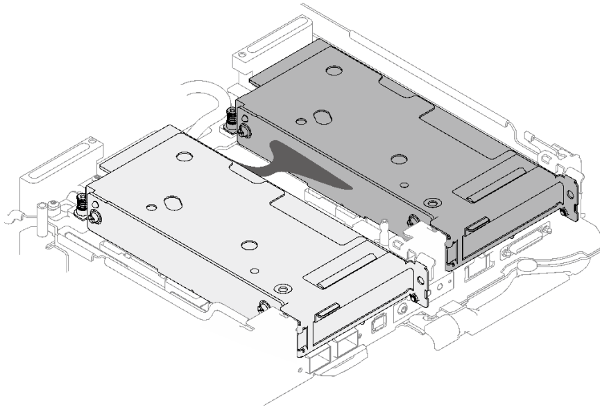
그림 155. 슬롯 1 및 슬롯 2에 설치되는 PCIe 라이저 유형
