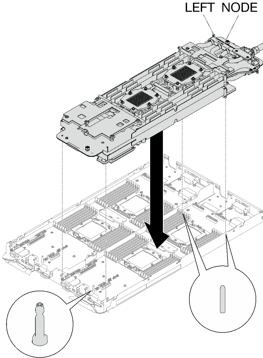
그림 27. 워터 루프 캐리어 설치
