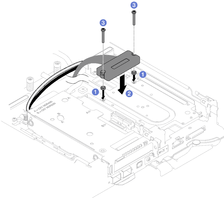
그림 177. 상호 연결 케이블 설치
