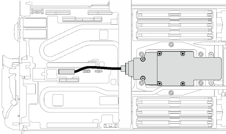
그림 128. M.2 백플레인 어셈블리 케이블 설치
