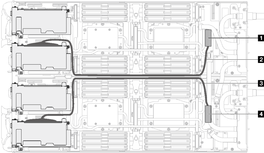
그림 282. 밸런스 I/O 구성
