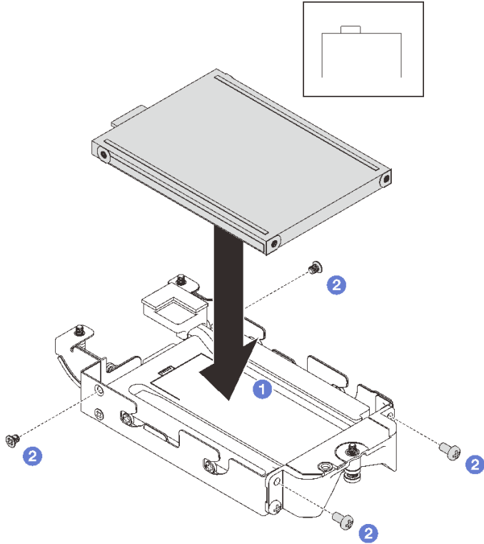
그림 109. 하단 E3.s 드라이브 설치
