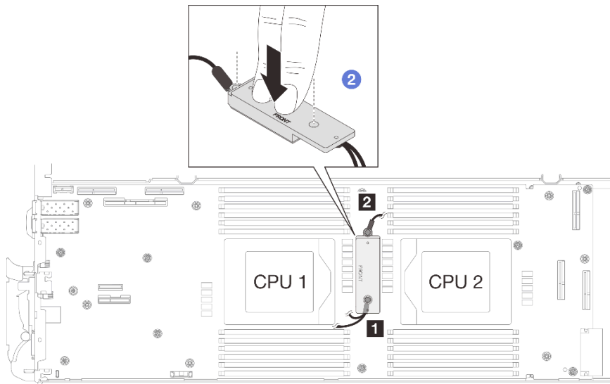
그림 254. VR 전도판 누르기
