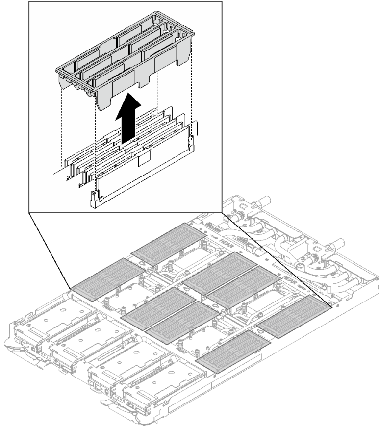
그림 131. DIMM 덮개 제거
