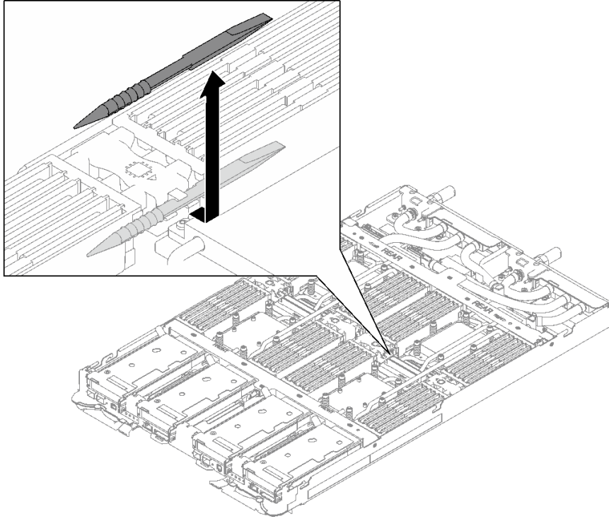
그림 130. 메모리 모듈 도구 제거
