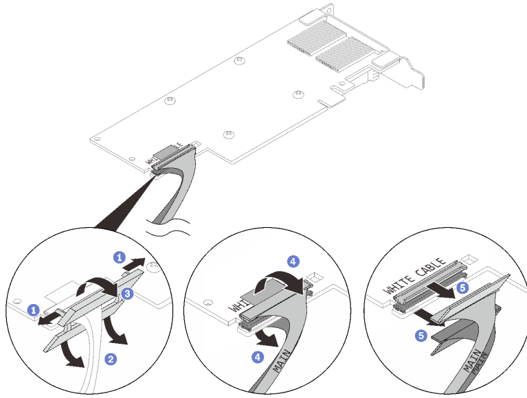
그림 144. PCIe 어댑터 케이블 제거
