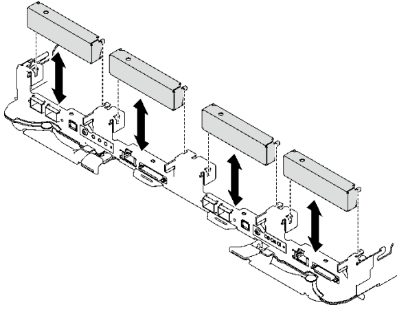
그림 153. 빈 베젤 필러 설치
