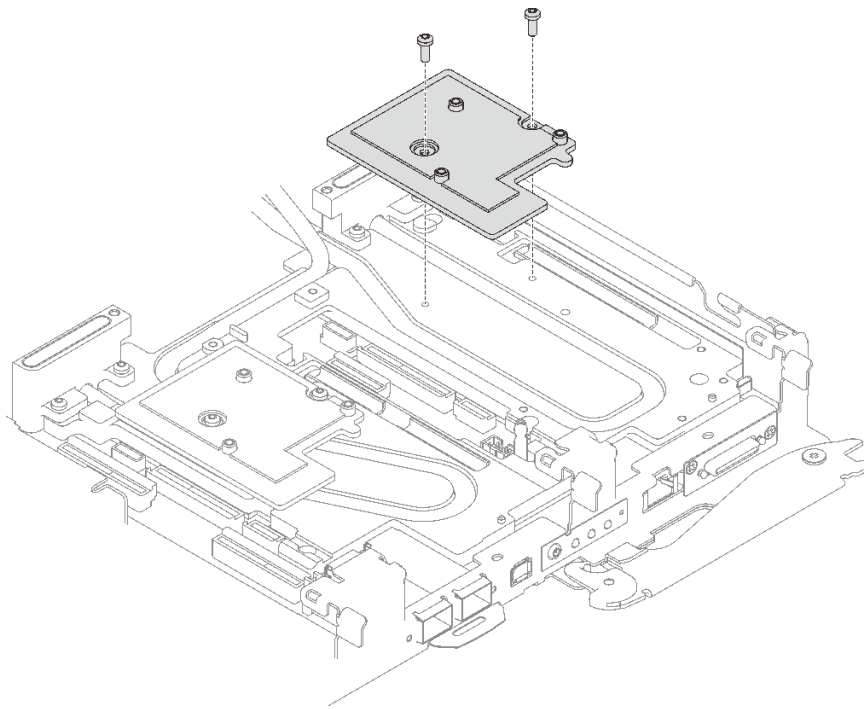
그림 190. 인터페이스판 설치
