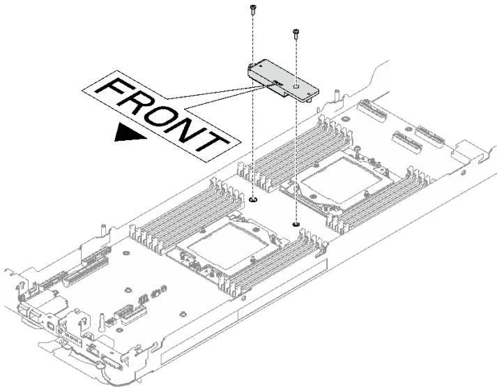
그림 279. VR 전도판 설치
