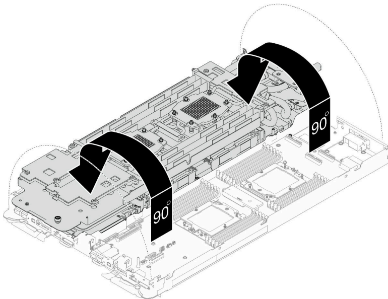
그림 226. 워터 루프 접기
