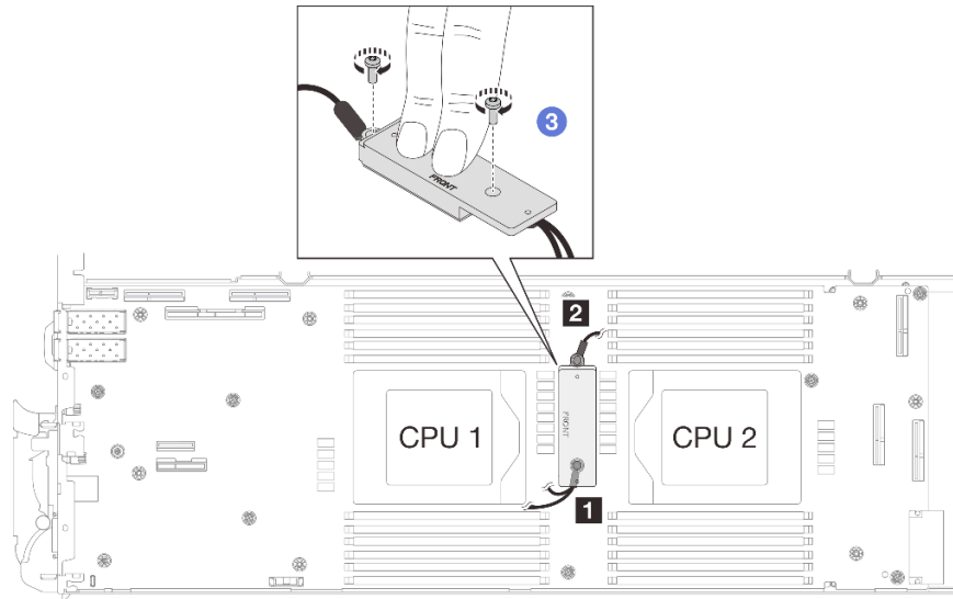
그림 255. 차폐 케이블 1/2 및 3 설치
