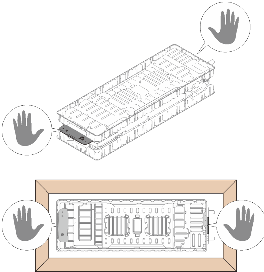
그림 21. 패키지 박스에서 워터 루프를 제거할 때의 터치 포인트
