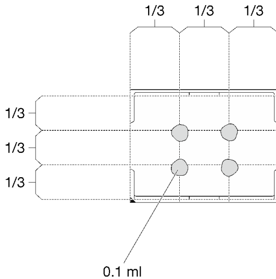
그림 205. 열전도 그리스 도포
