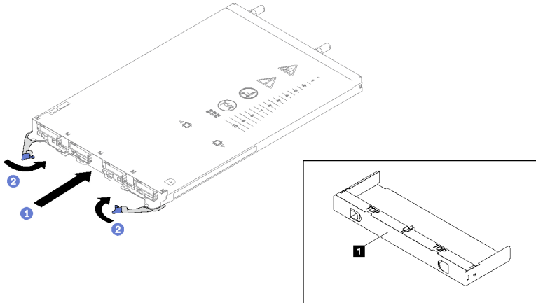
그림 5. 트레이 설치
