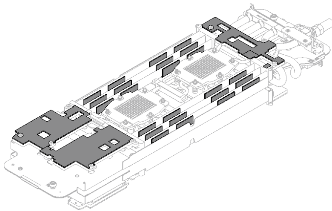
그림 232. 워터 루프 캡 패드(하단)
