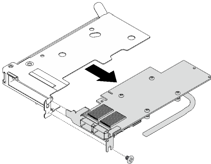
그림 143. PCIe 어댑터 제거
