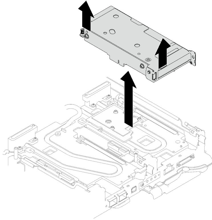
그림 181. PCIe 라이저 케이스 어셈블리 제거
