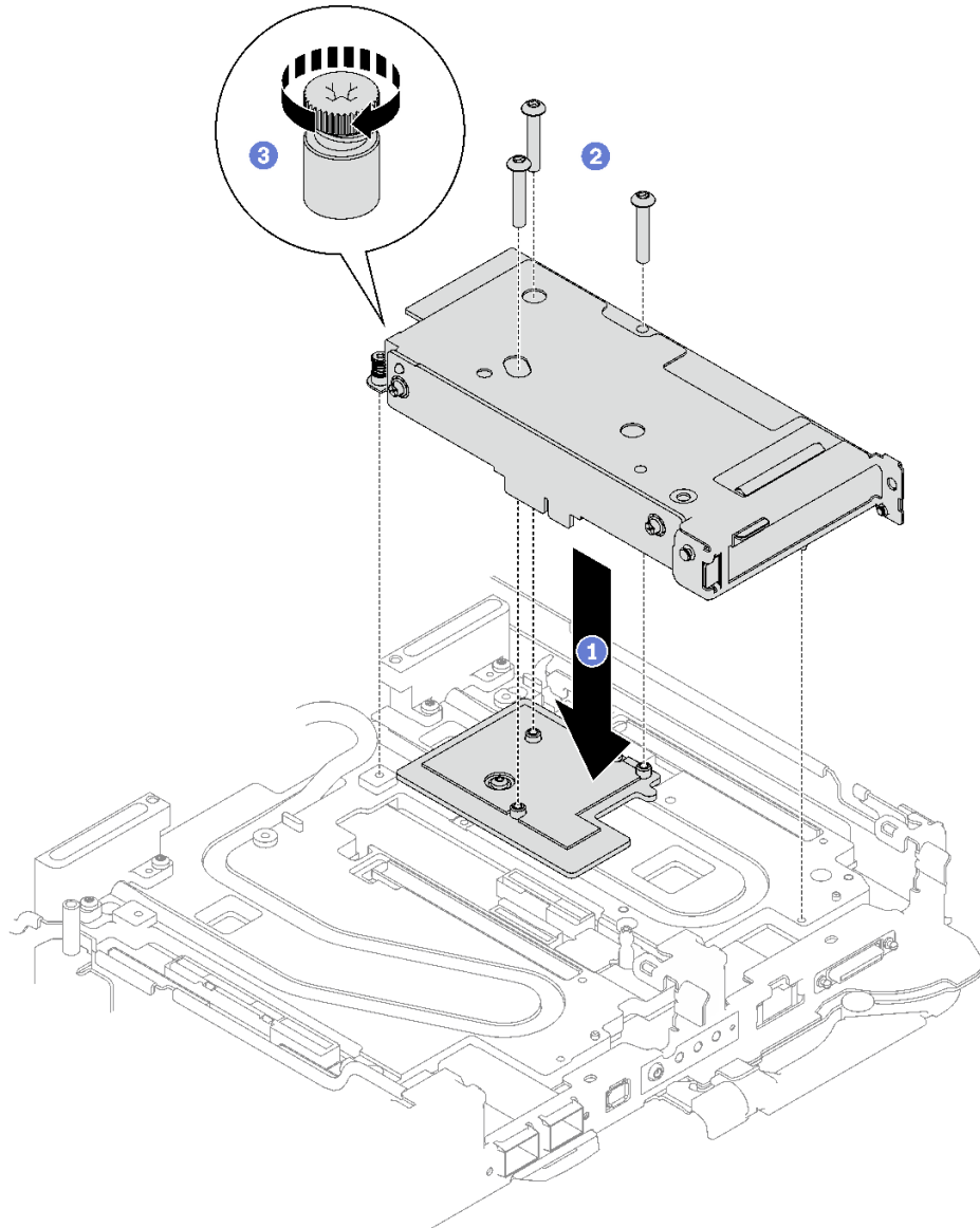
그림 192. PCIe 라이저 어셈블리 설치
