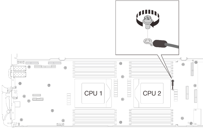
그림 257. 차폐 케이블 4 설치
