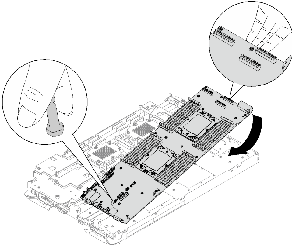
그림 269. 시스템 보드 설치
