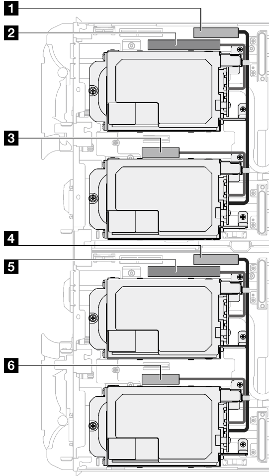
그림 117. E3.s 드라이브 케이블 배선
