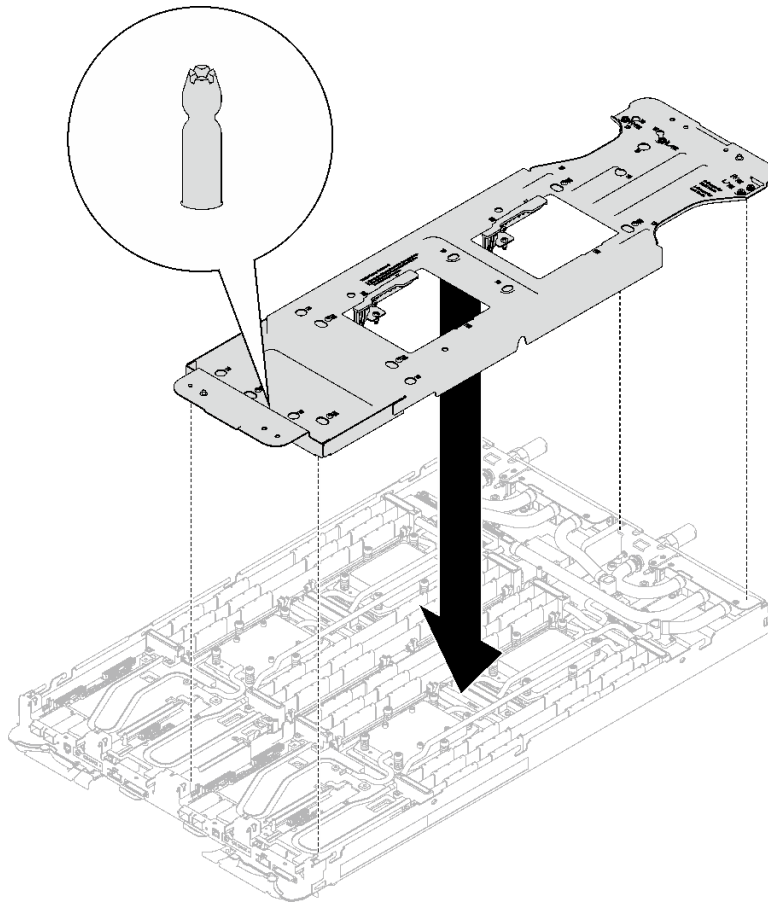
그림 221. 워터 루프 캐리어 설치
