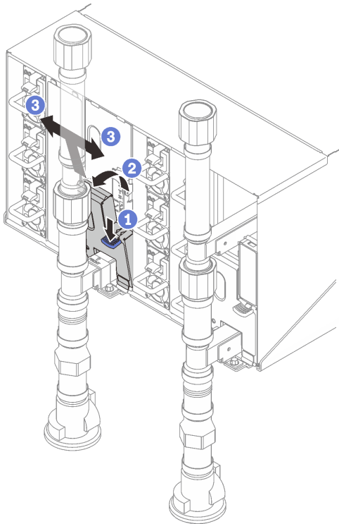
그림 295. 하단 EMC 실드 제거
