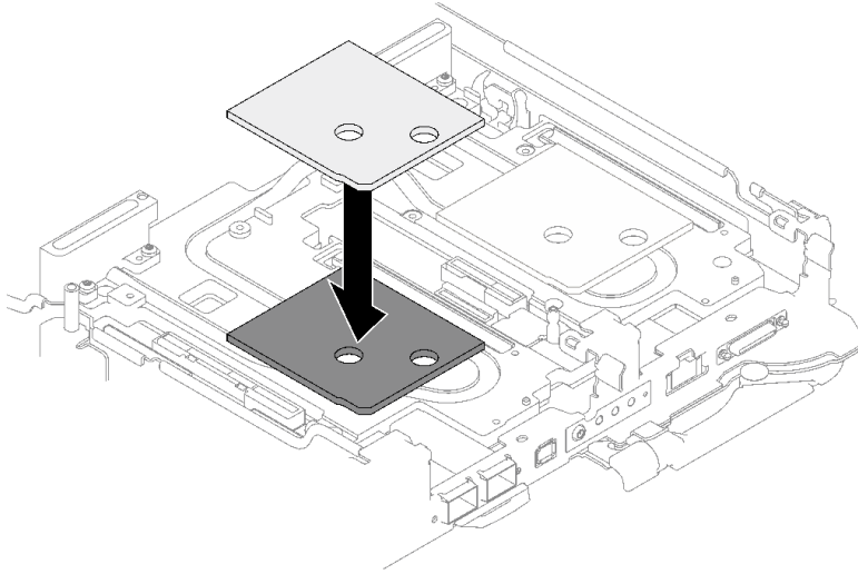
그림 74. 겹 패드 교체
