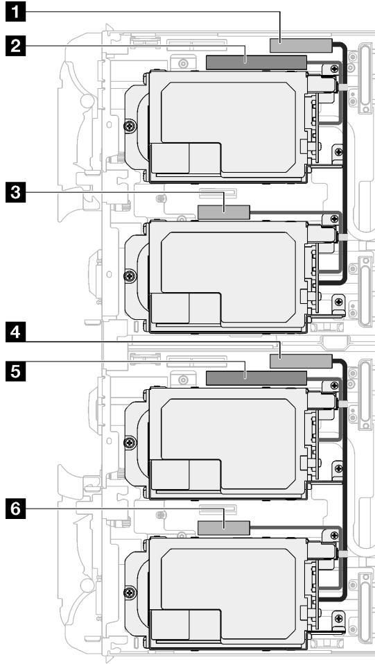
그림 96. E3.s 드라이브 케이블 배선
