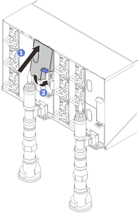
그림 297. 상단 EMC 실드 설치
