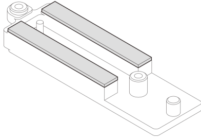
그림 44. VR 전도판 하단의 퍼티 패드
