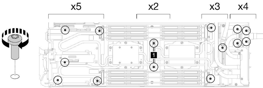
그림 34. 워터 루프 나사 및 퀵 커넥트 나사 설치
