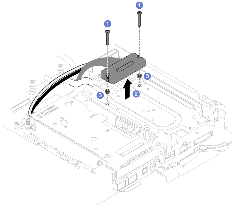
그림 178. 상호 연결 케이블 제거
