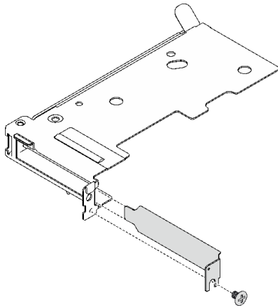
그림 145. 필러 설치
