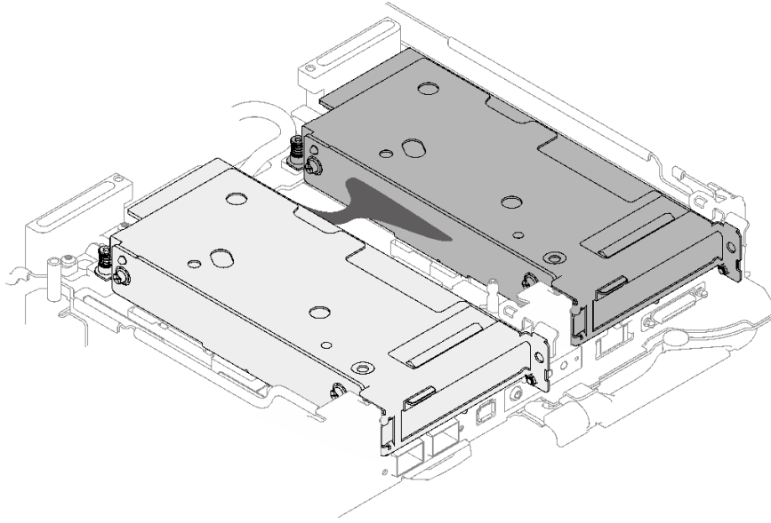
그림 171. 슬롯 1 및 슬롯 2에 설치되는 PCIe 라이저 유형
