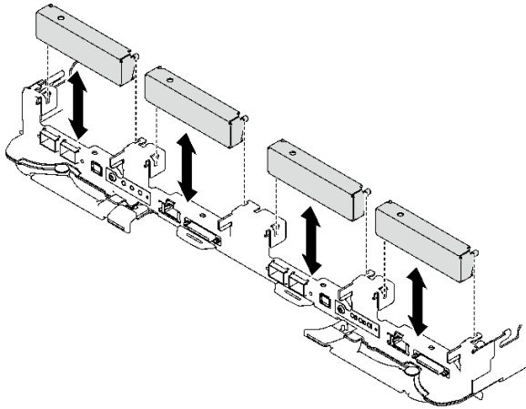
그림 98. 빈 베젤 필터 제거
