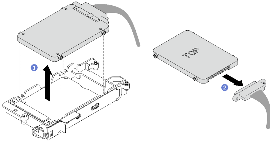
그림 63. 하단 드라이브 제거
