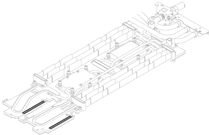
그림 25. 워터 루프 갭 패드(상단)
