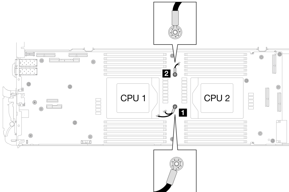
그림 39. 차폐 케이블 1/2 및 차폐 케이블 3을 나사 구멍에 맞추기
