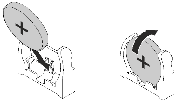
그림 49. CMOS 배터리 설치
