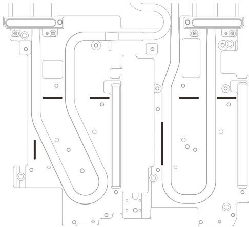
그림 73. 겹 패드를 맞추기 위한 워터 루프의 표시
