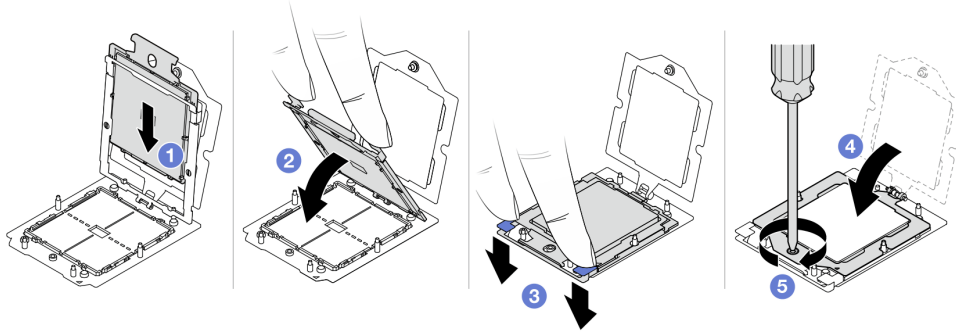
그림 229. 프로세서 설치
