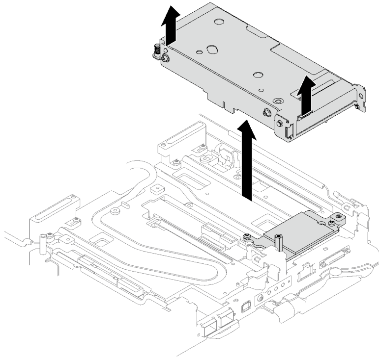
그림 151. PCIe 라이저 어셈블리 풀기
