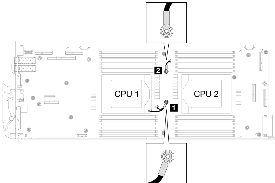
그림 252. 차폐 케이블 1/2 및 차폐 케이블 3을 나사 구멍에 맞추기
