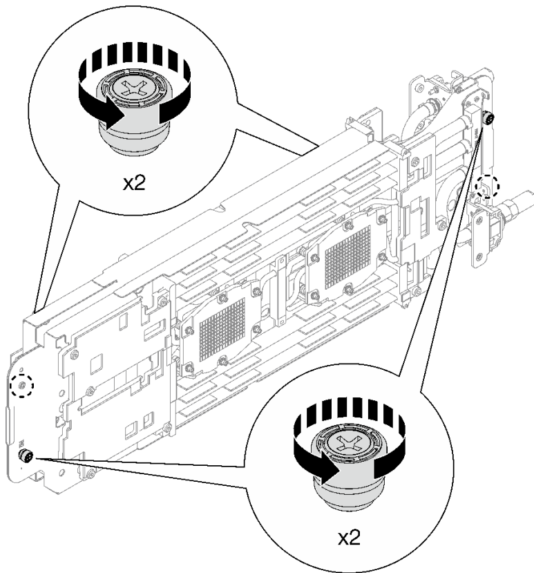
그림 23. 워터 루프 캐리어 고정 나비 나사 풀기
