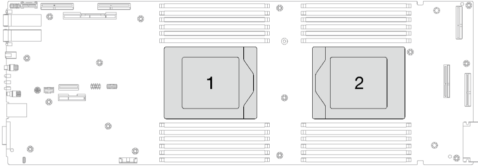
그림 228. 프로세서 위치
