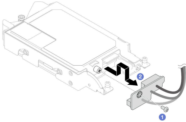
그림 101. E3.s 드라이브 케이블 종단 백플레인 제거
