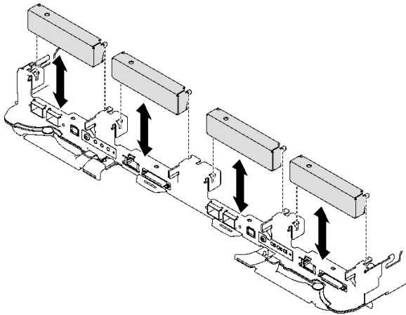
그림 169. 빈 베젤 필터 설치
