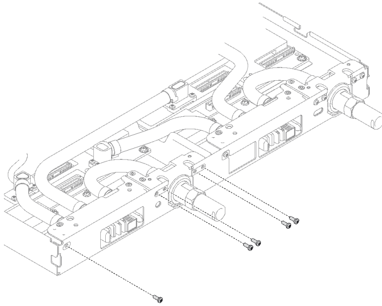
그림 216. 클릭 커넥트 나사 설치
