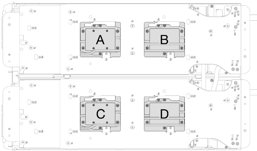
그림 30. 프로세서 냉각판 설치
