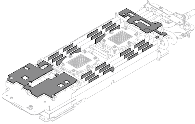
그림 24. 워터 루프 갭 패드(하단)
