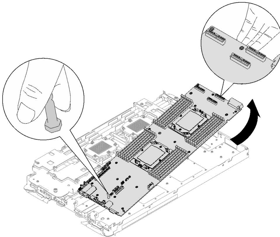
그림 246. 시스템 보드 제거
