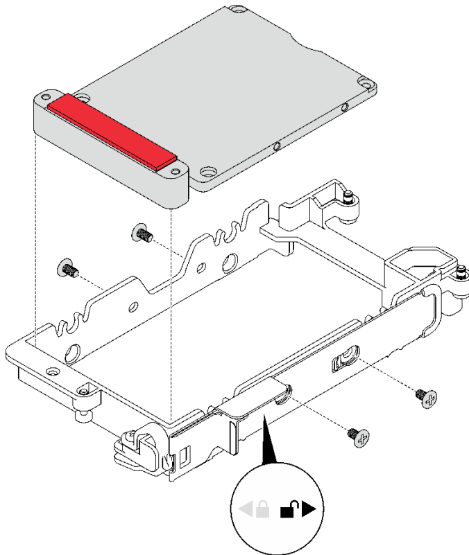
그림 64. 전도판 제거
