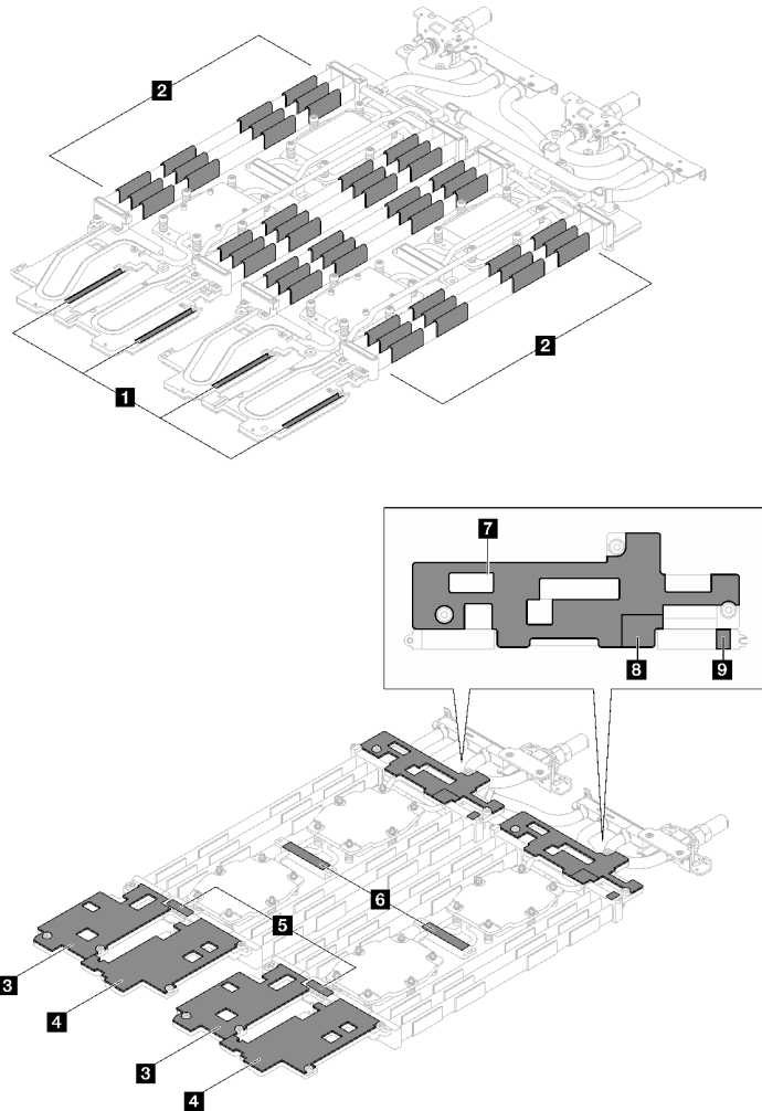
그림 2. 위터 루프 - 갭 패드/퍼티 패드 식별 및 위치
