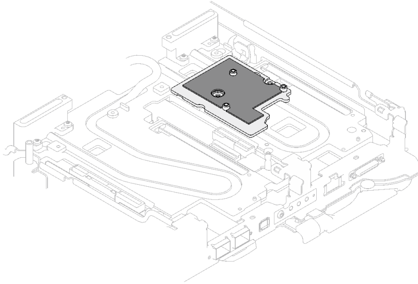
그림 191. CX-7 NDR 400용 인터페이스판의 갭 패드
