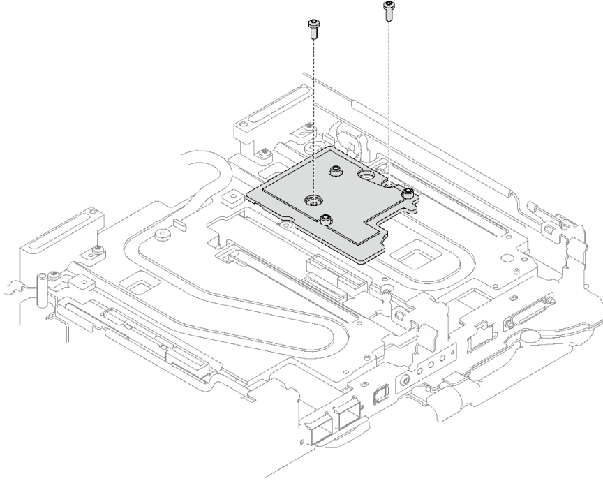
그림 182. 인터페이스판 제거
