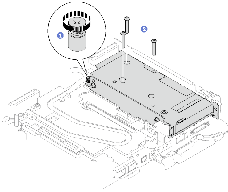
그림 179. PCIe 라이저 어셈블리 제거
