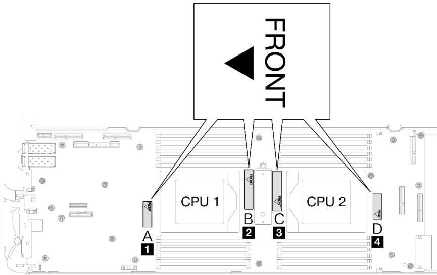
그림 262. 앞면을 가리키는 케이지의 앞면 표시
