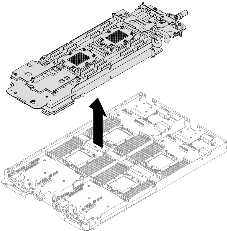
그림 20. 워터 루프 제거
