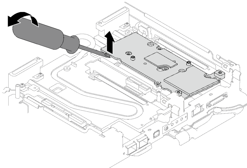
그림 167. 워터 루프 냉각판에서 인터페이스판 분리
