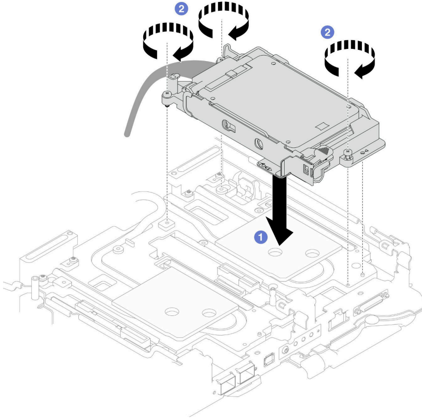
그림 94. 7mm NVMe 드라이브 케이지 어셈블리 설치
