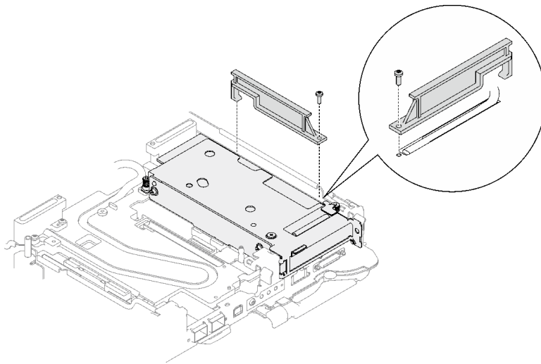
그림 161. 히트파이프 빔 설치
