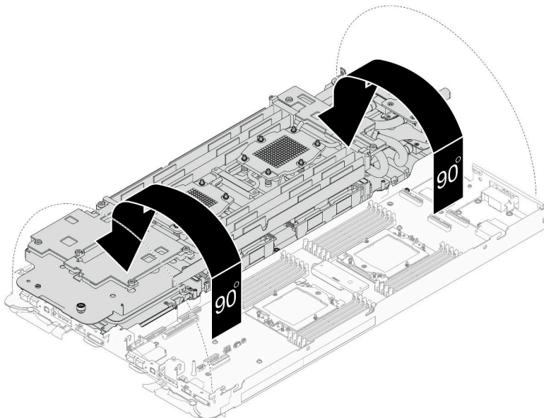
그림 202. 워터 루프 접기
