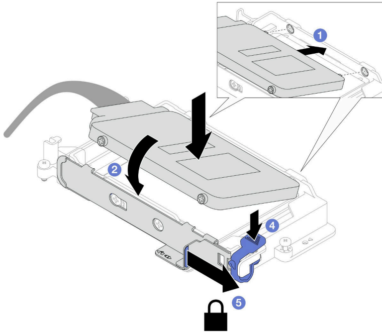
그림 89. 위쪽 드라이브 설치
