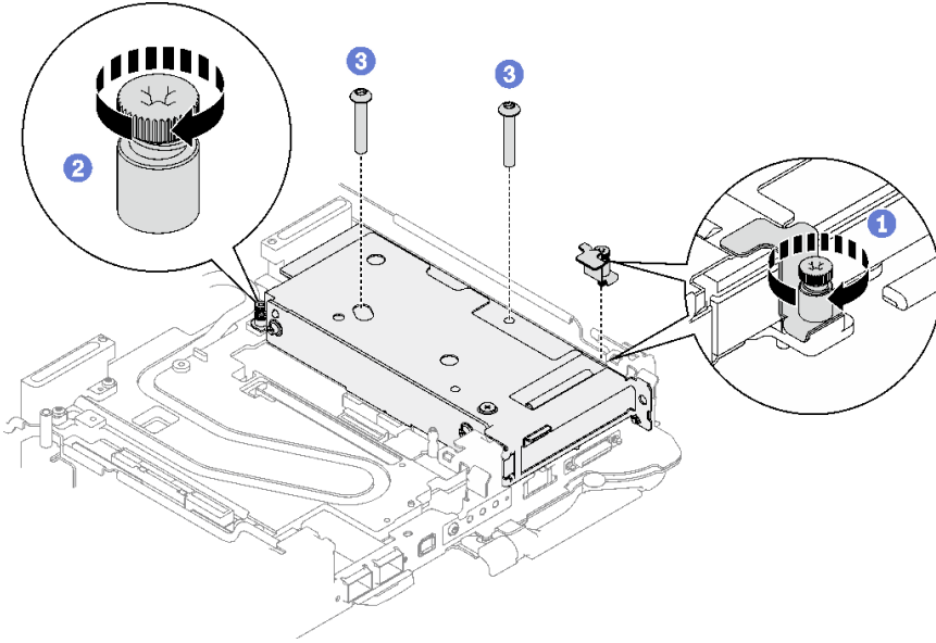
그림 176. 클램프 브래킷 고정 나사 설치
