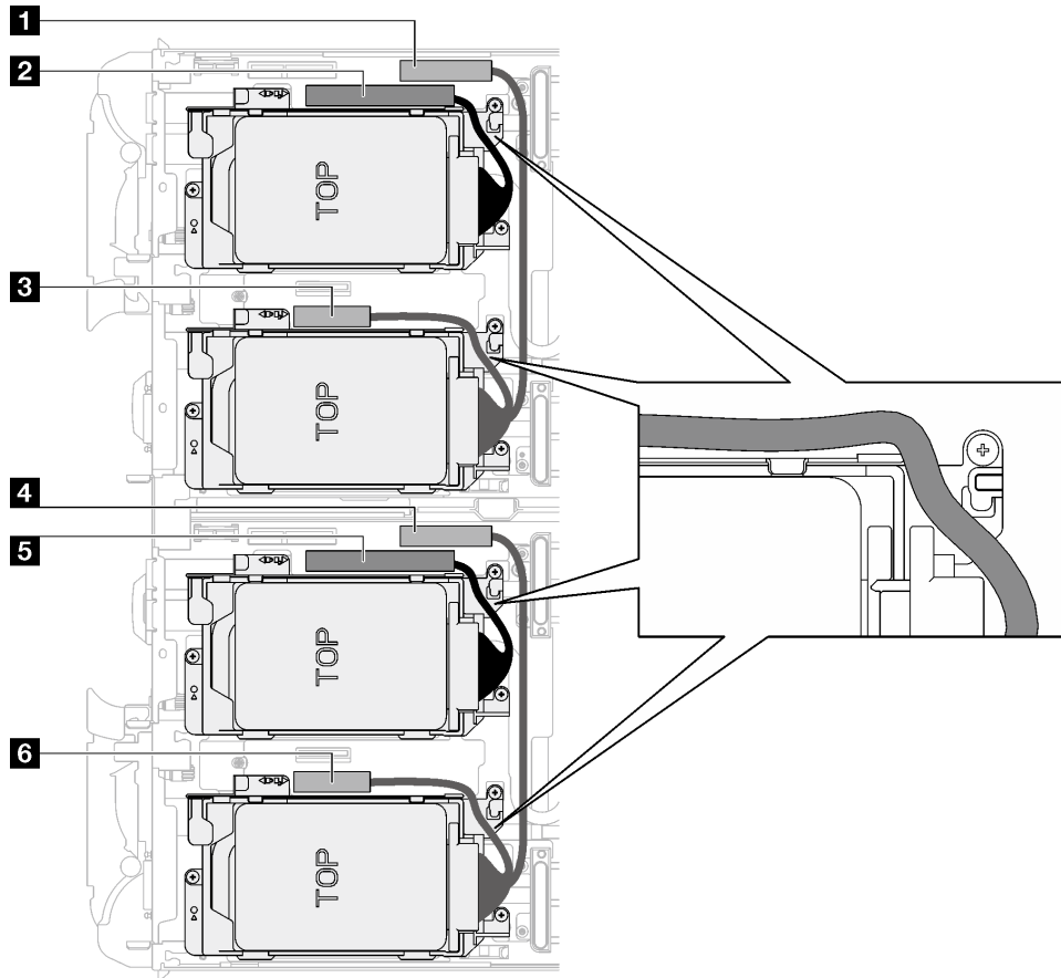
그림 81. 모든 NVMe 드라이브용 드라이브 어셈블리 케이블 배선
