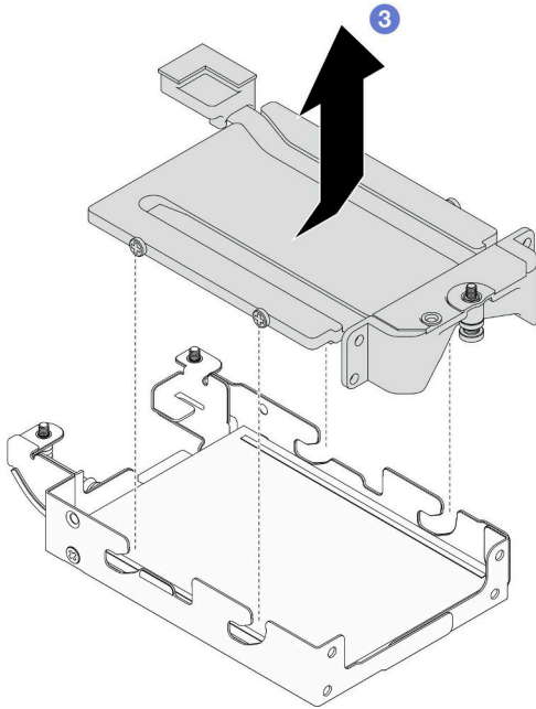
그림 103. 전도판 제거
