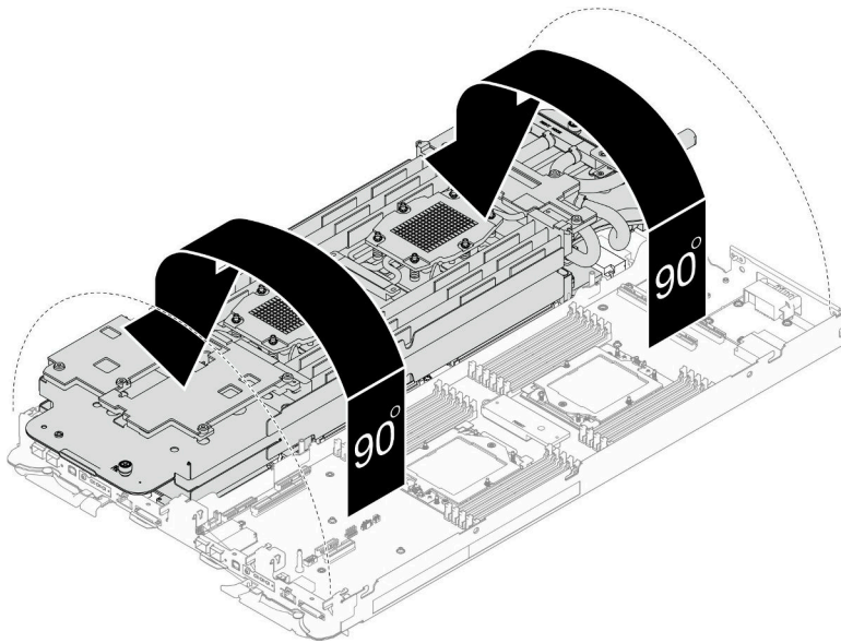
그림 18. 워터 루프 접기
