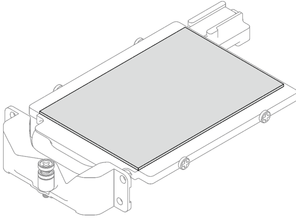
그림 106. 전도판 갭 패드 교체
