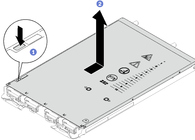
그림 6. 트레이 덮개 제거
