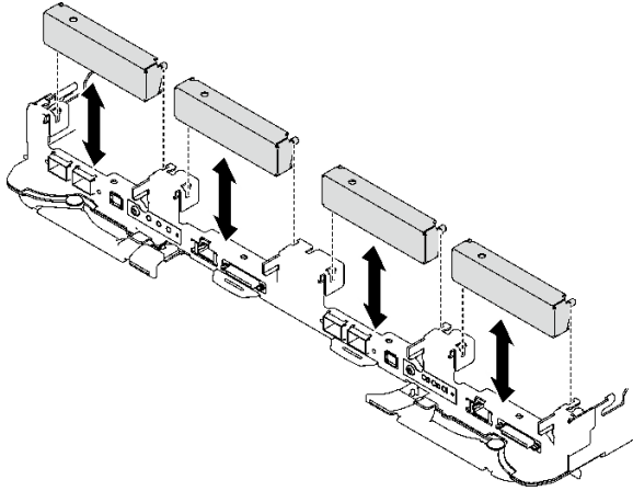
그림 90. 빈 베젤 필러 설치
