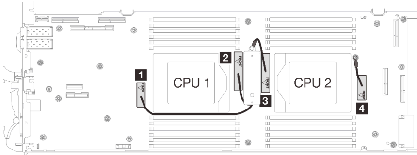
그림 265. 차폐 케이시의 케이블 배선
