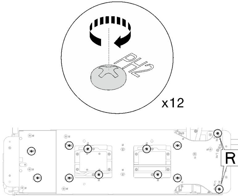
그림 198. 워터 루프 캐리어 나사 설치
