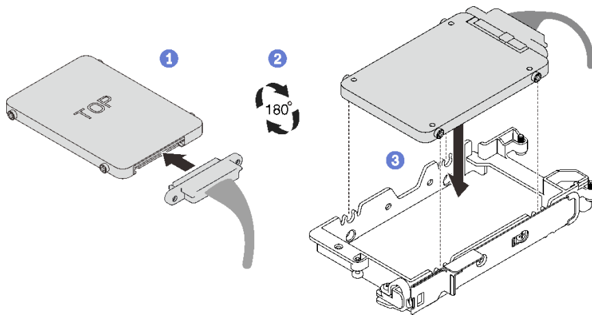
그림 69. 아래쪽 드라이브 설치
