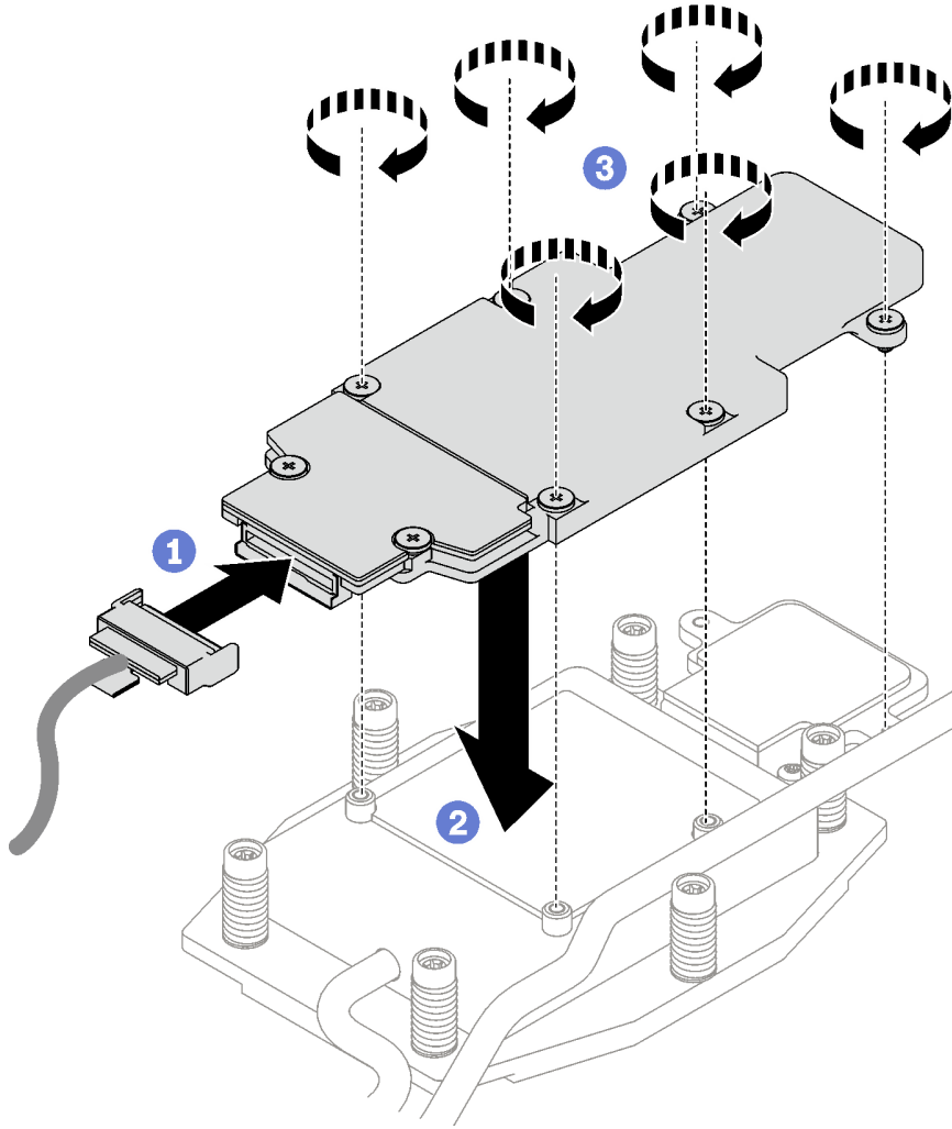
그림 127. M.2 백플레인 어셈블리 설치
