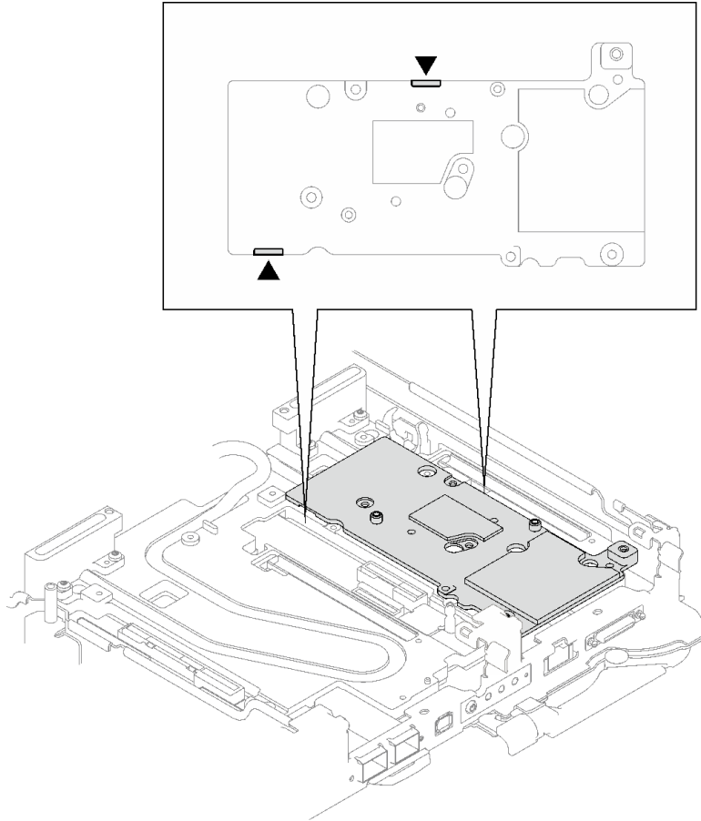
그림 166. 인터페이스판 하단의 구멍 위치
