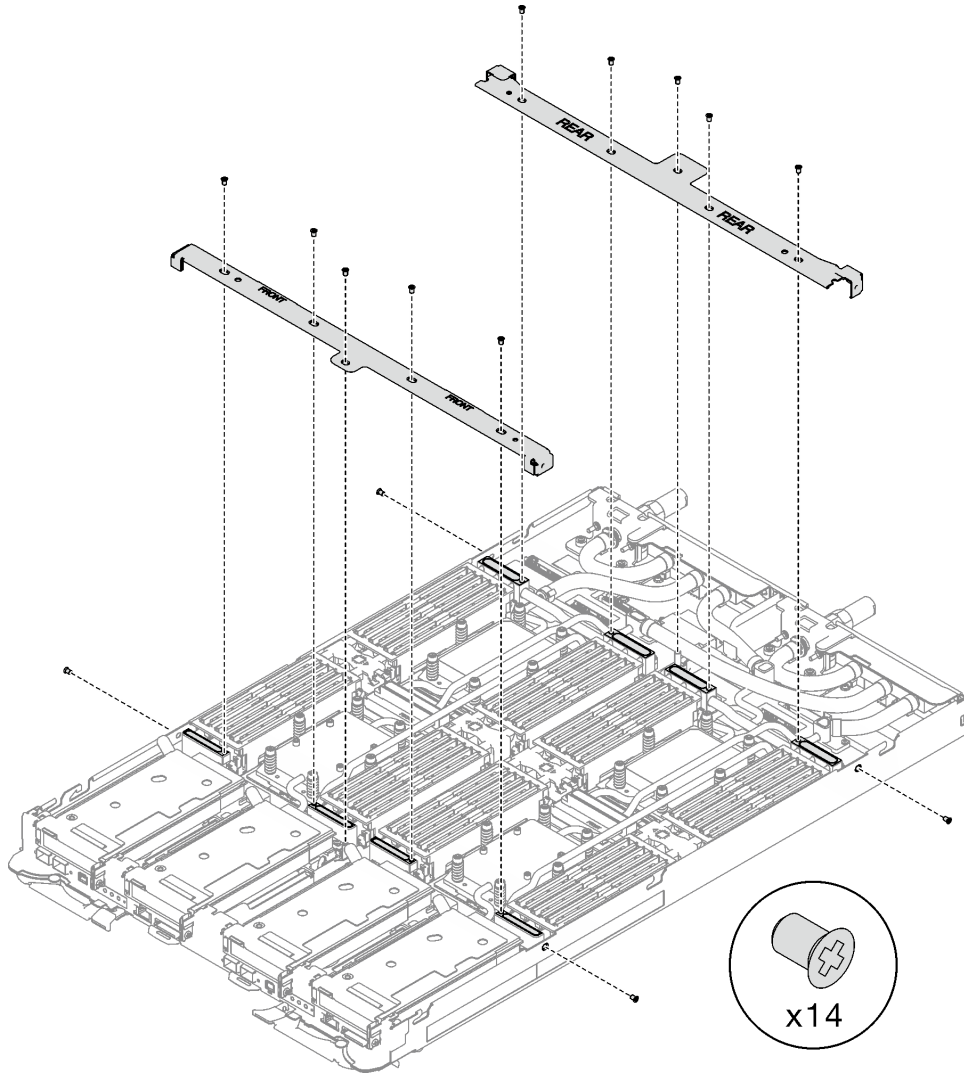
그림 9. 십자형 브레이스 설치
