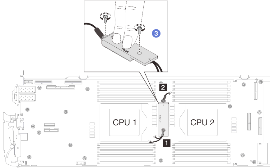
그림 42. 차폐 케이블 1/2 및 3 설치
