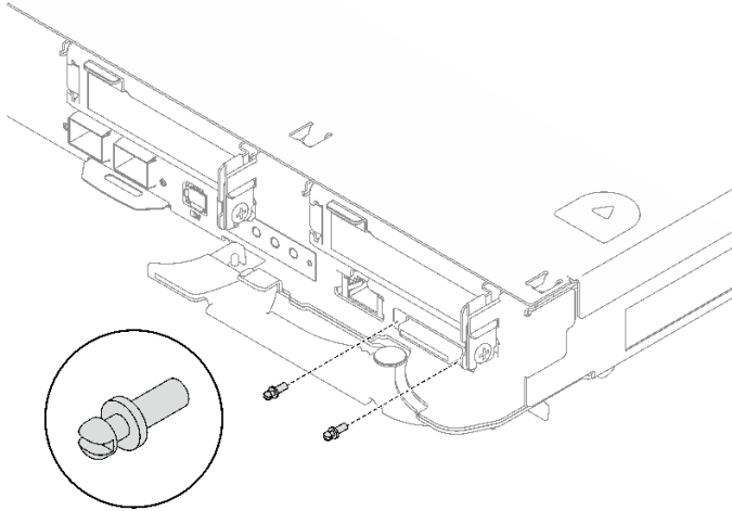
그림 243. KVM 나사 제거
