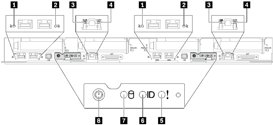
그림 288. SD665 V3 트레이 앞면 LED
