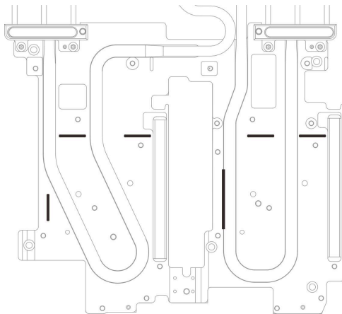
그림 91. 갭 패드를 맞추기 위한 워터 루프의 표시
