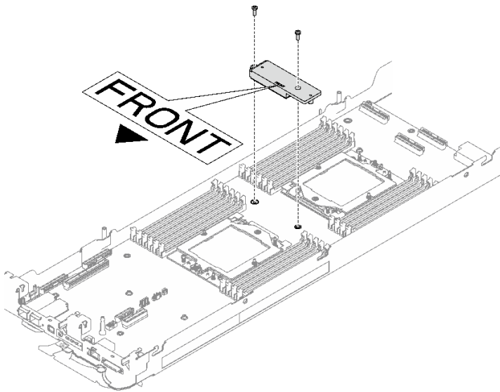
그림 244. VR 전도판 제거
