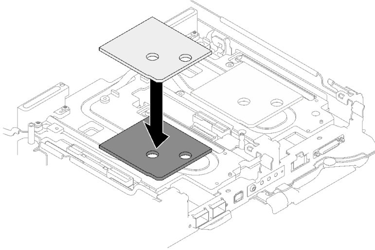
그림 92. 겹 패드 교체
