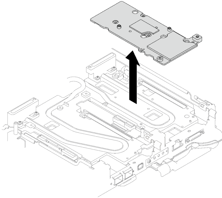
그림 168. 인터페이스판 제거
