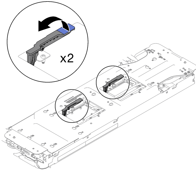
그림 201. 프로세서에서 워터 루프 분리
