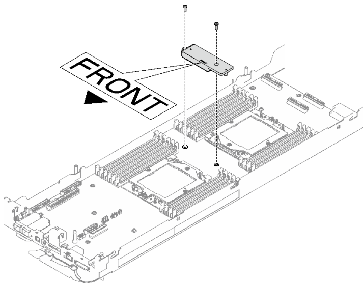
그림 45. VR 전도판 제거
