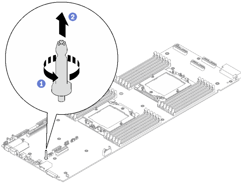
그림 247. 가이드 핀 제거
