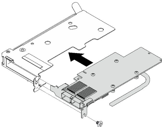
그림 148. PCIe 어댑터 설치
