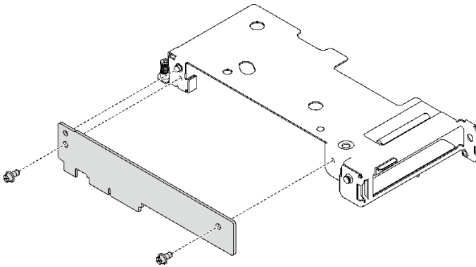
그림 154. 확장 보드 제거
