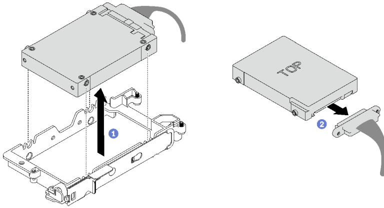
그림 61. 15mm 드라이브 제거
