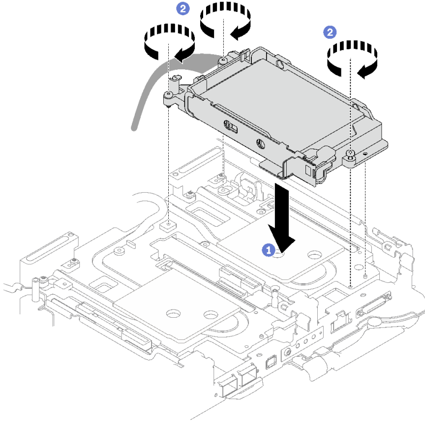
그림 78. 15mm 드라이브 케이지 어셈블리 1개 설치
