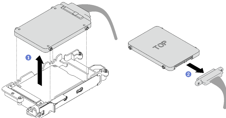
그림 60. 7mm 드라이브 제거
