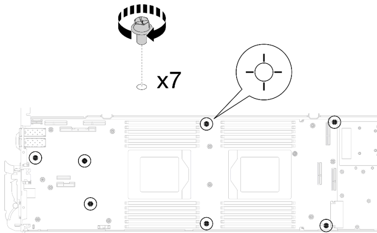
그림 266. 시스템 보드 나사 설치
