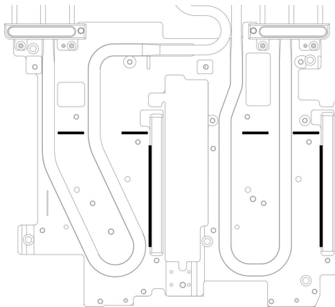
그림 114. E3.S 갭 패드를 맞추기 위한 워터 루프의 표시
