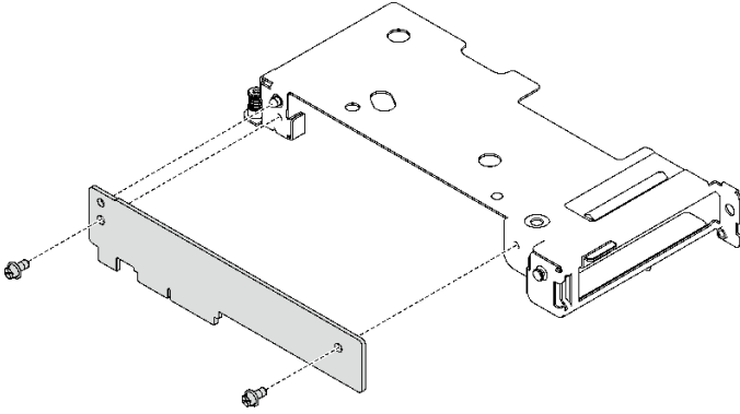
그림 187. 확장 보드 제거
