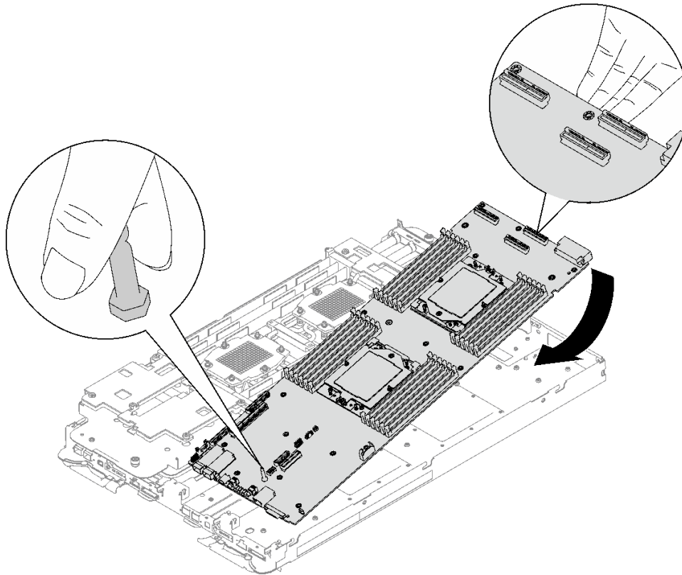
그림 249. 시스템 보드 설치
