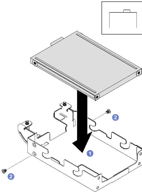
그림 105. 상단 E3.s 드라이브 설치
