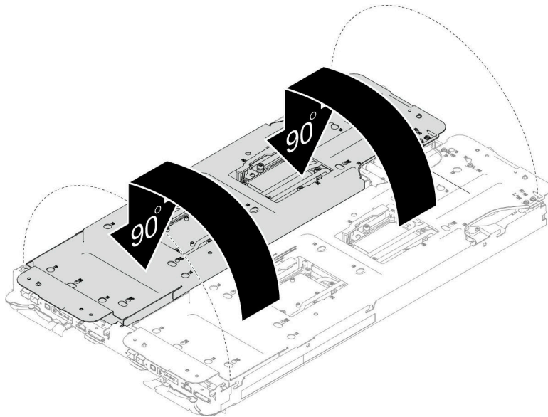
그림 29. 워터 루프 펼치기
