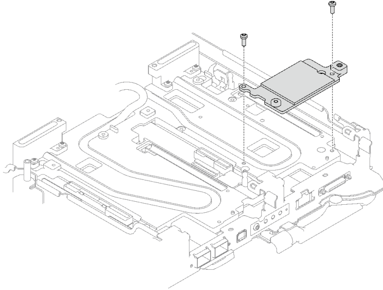
그림 157. 인터페이스판 설치
