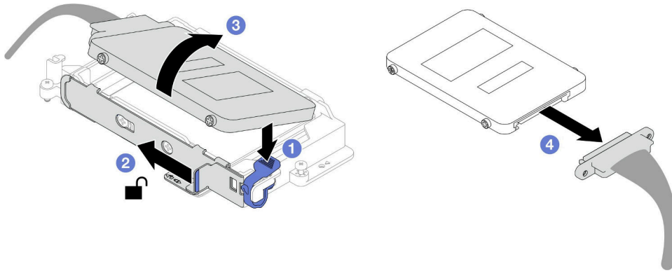
그림 84. 상단 드라이브 제거(7mm NVMe)
