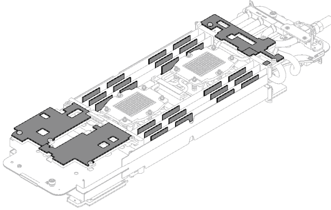
그림 206. 워터 루프 캡 패드(하단)
