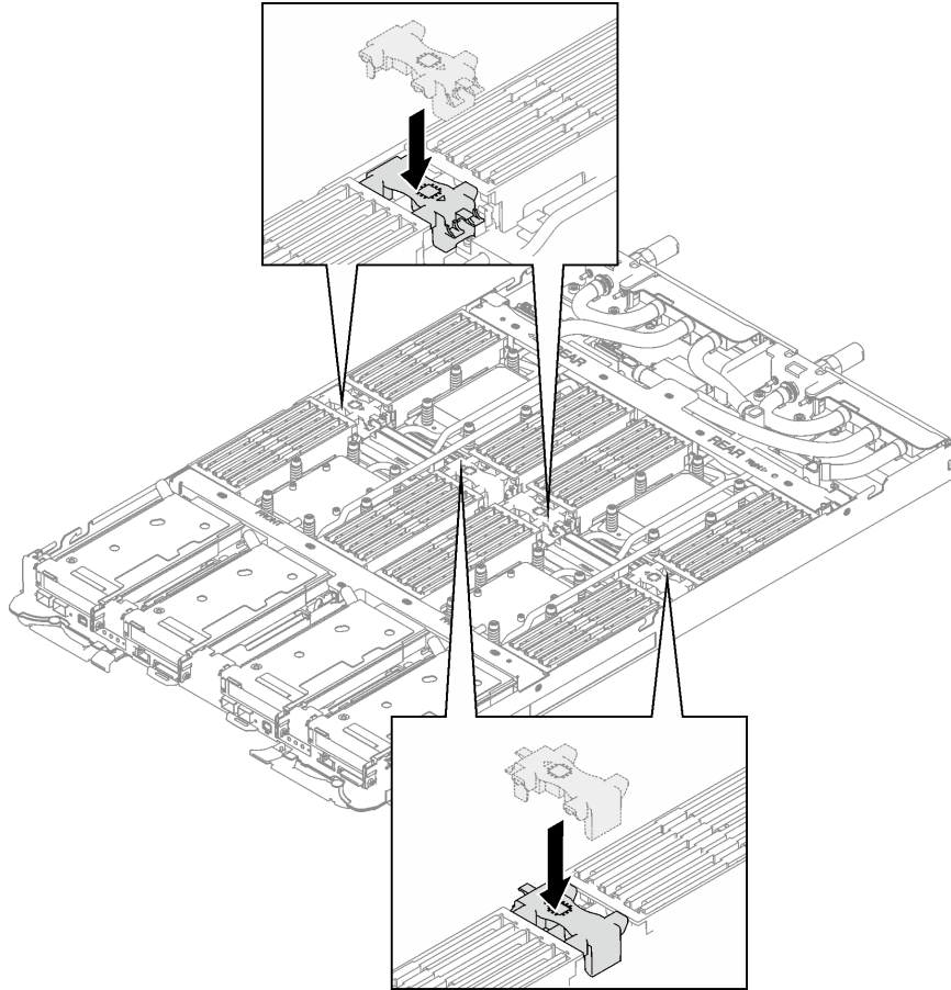
그림 52. DIMM 콤 설치
