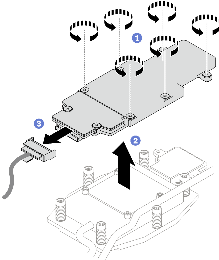
그림 119. M.2 백플레인 어셈블리 제거
