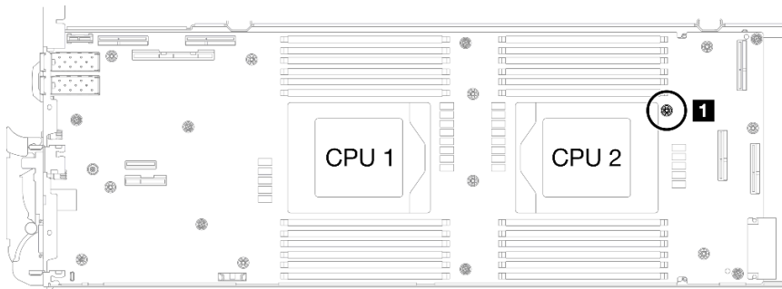
그림 256. 차폐 케이블 4의 나사 구멍 위치
