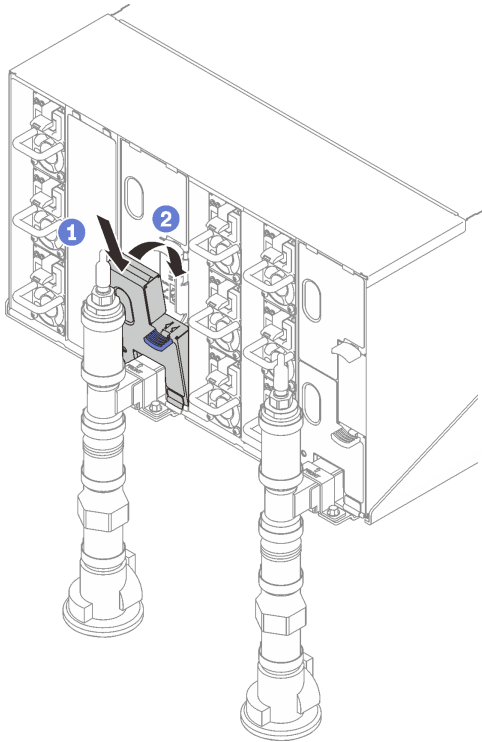
그림 298. 하단 EMC 실드 설치
