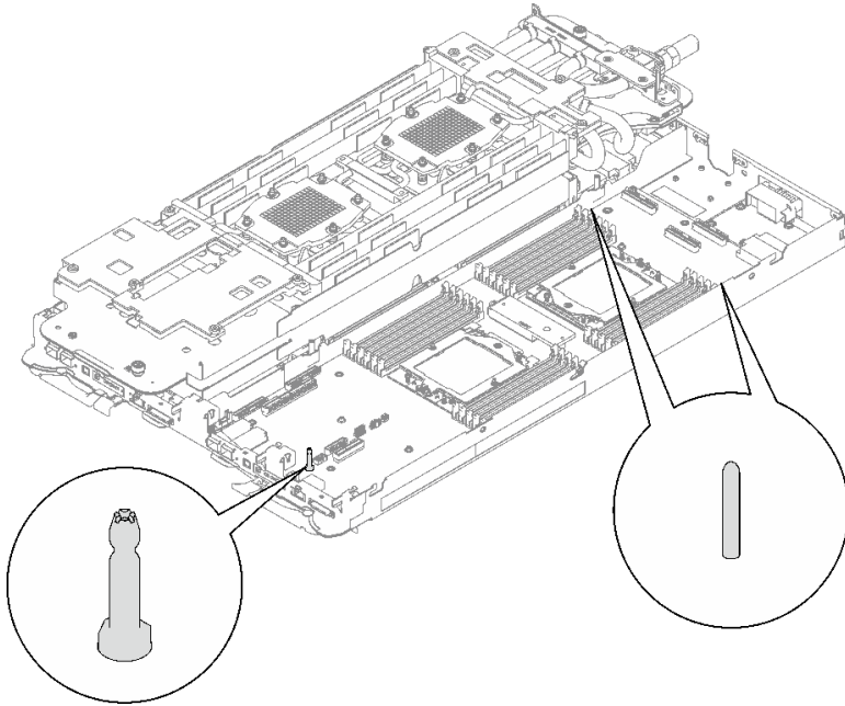
그림 209. 오른쪽 컴퓨팅 노드의 가이드 핀
