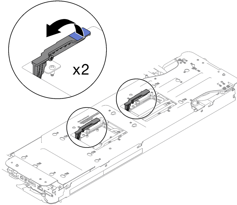
그림 225. 프로세서에서 워터 루프 분리
