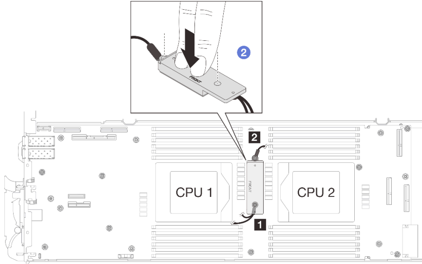
그림 271. VR 전도판 누르기
