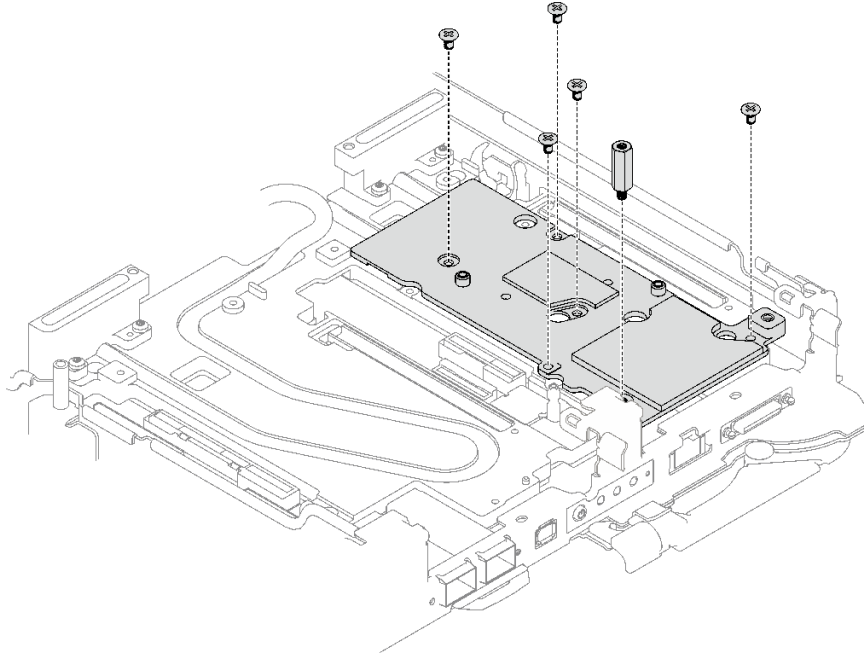
그림 165. 인터페이스판 나사 제거
