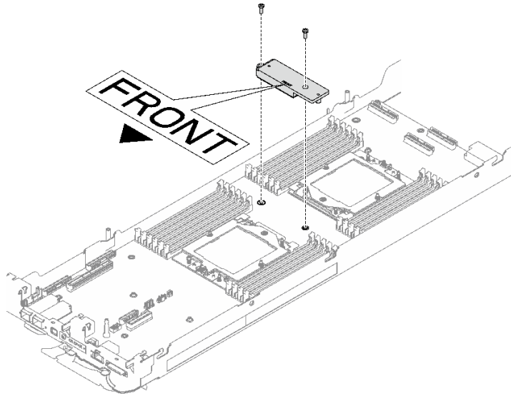
그림 36. VR 전도판 제거
