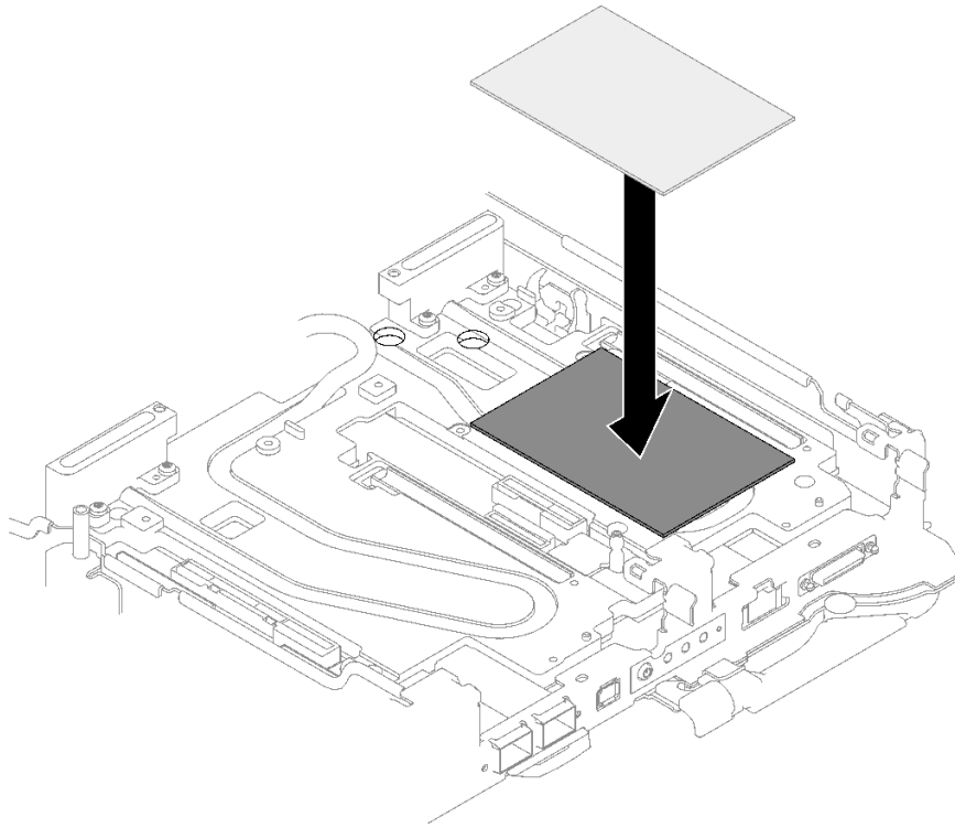
그림 115. 캡 패드 교체
