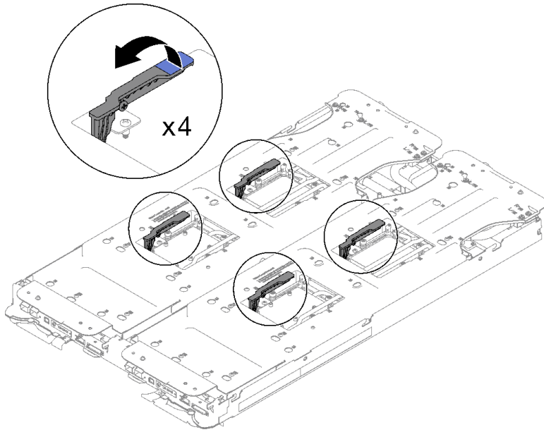
그림 17. 프로세서에서 워터 루프 분리
