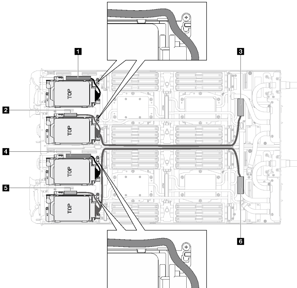
그림 54. SATA 드라이브용 드라이브 어셈블리 케이블 배선
