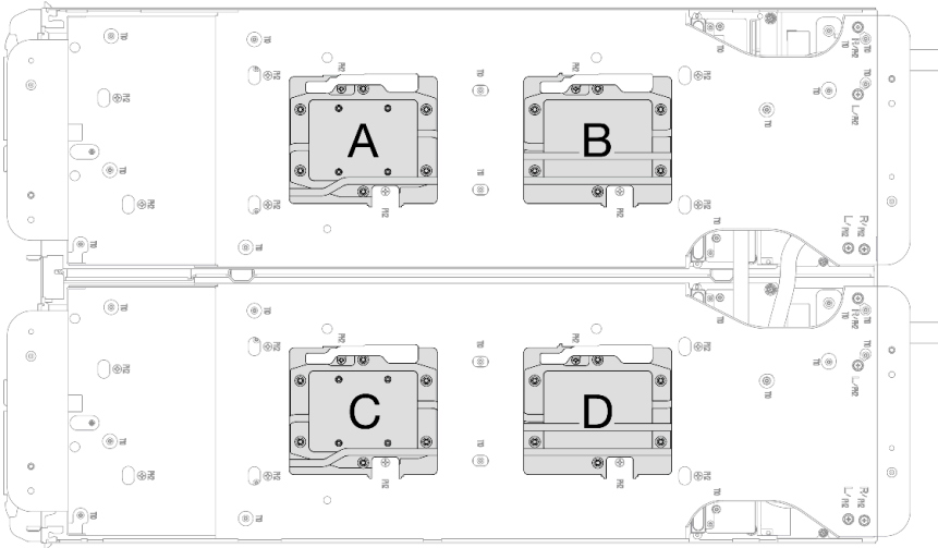
그림 211. 프로세서 냉각판 설치
