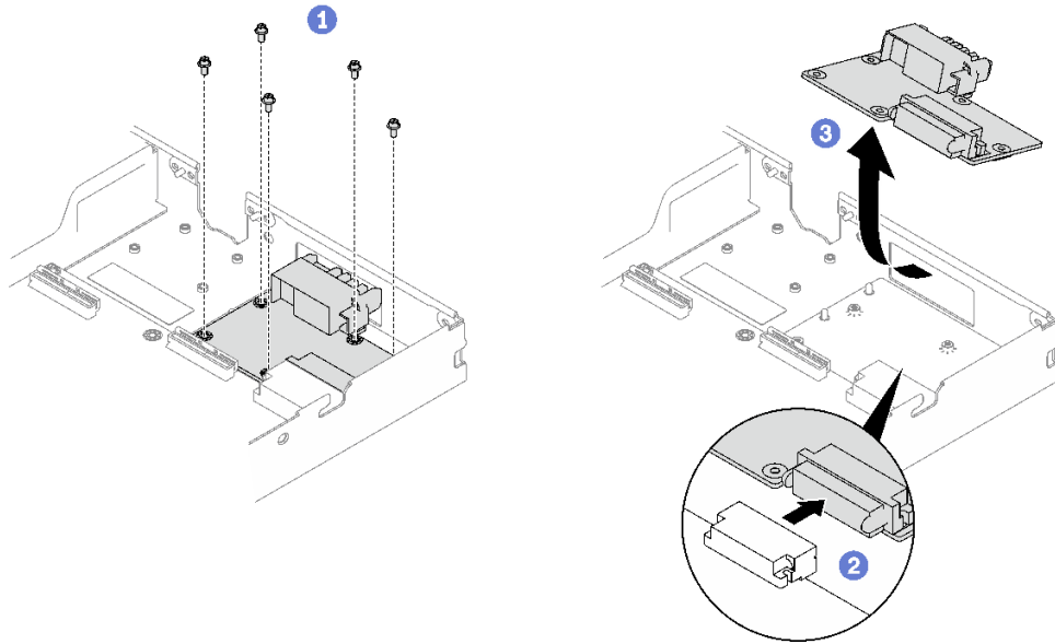
그림 203. 전원 분배 보드 제거
