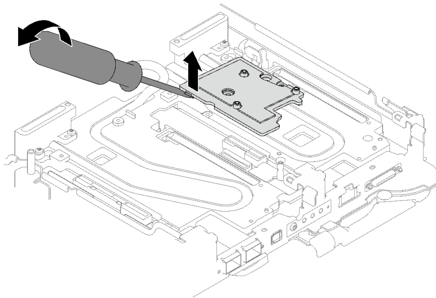
그림 184. 워터 루프 냉각판에서 인터페이스판 분리
