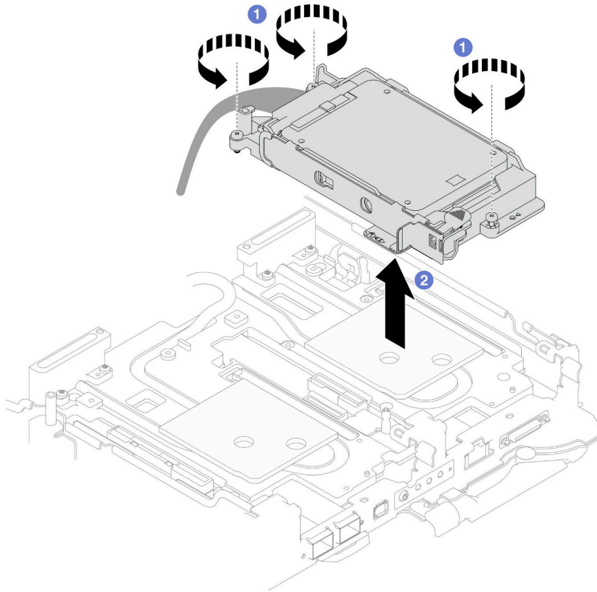
그림 82. 7mm NVMe 드라이브 케이스 어셈블리 제거
