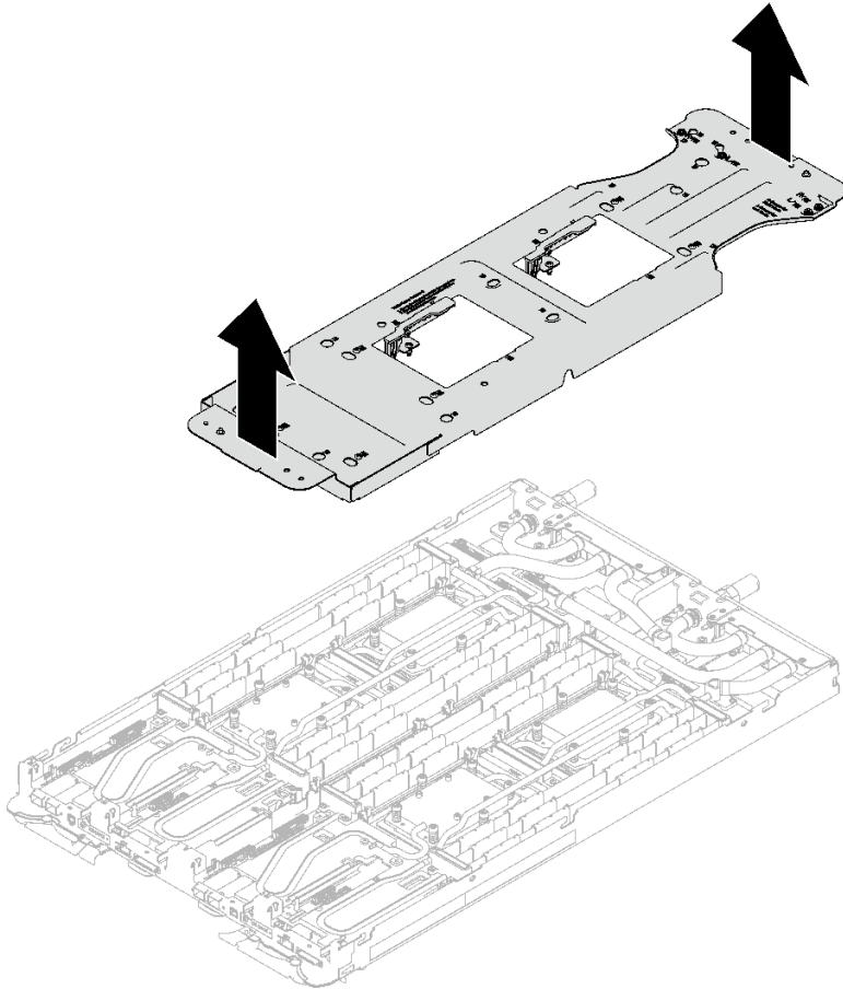
그림 213. 워터 루프 캐리어 제거
