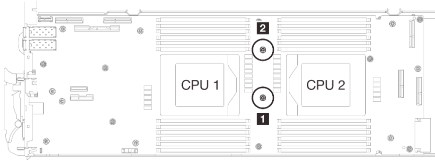
그림 38. 차폐 케이블 1/2 및 3의 나사 구멍 위치
