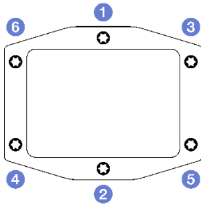
그림 223. 프로세서 냉각판 레이블
