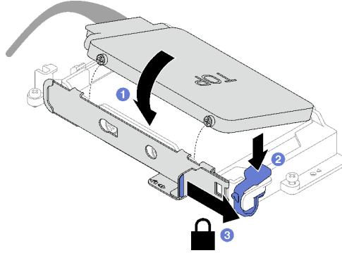
그림 70. 위쪽 드라이브 설치
