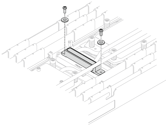
그림 219. 와셔가 있는 VR 냉각판 나사
