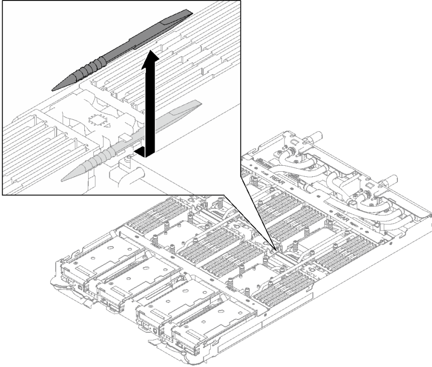
그림 137. 메모리 모듈 도구 제거
