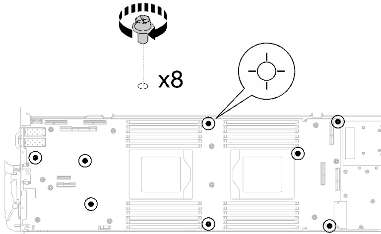
그림 245. 시스템 보드 나사 제거
