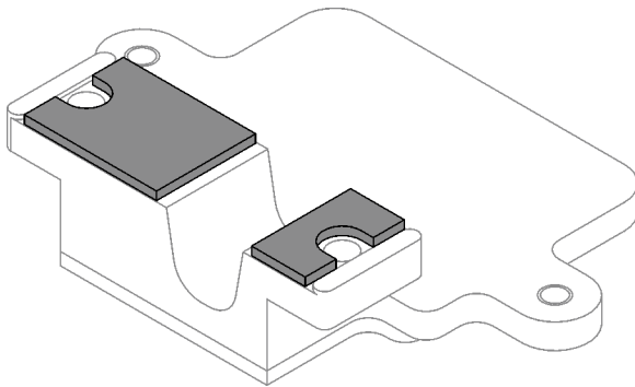
그림 124. M.2 백플레인 냉각판의 퍼티 패드(하단)
