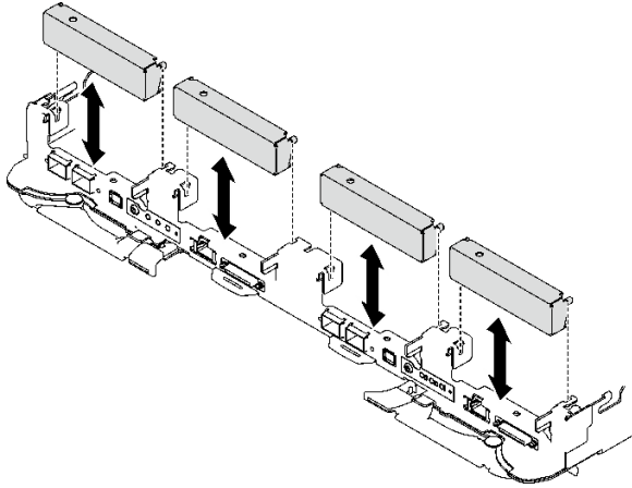
그림 189. 빈 베젤 필터 제거
