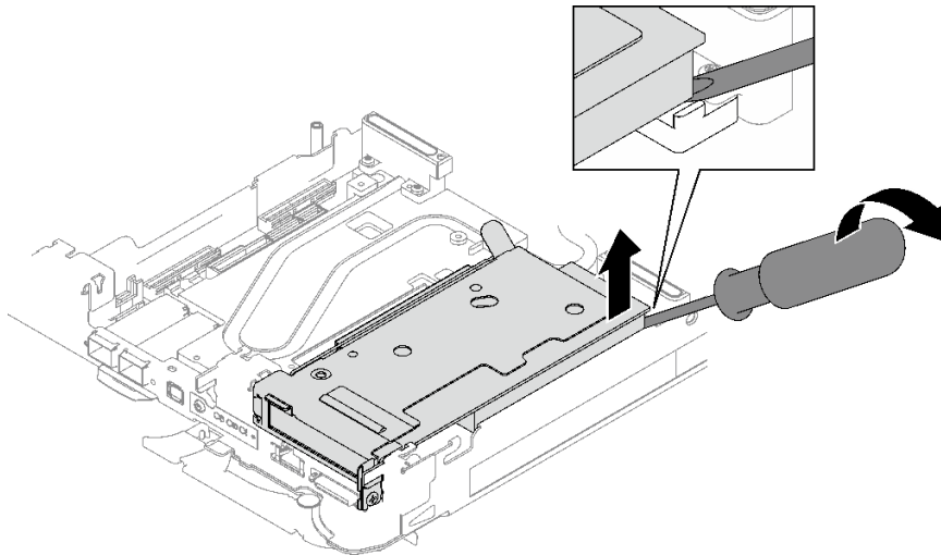
그림 180. 워터 루프 냉각판에서 PCIe 라이저 케이스 분리
