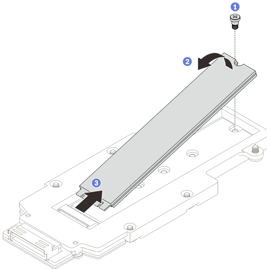
그림 121. M.2 드라이브 제거
