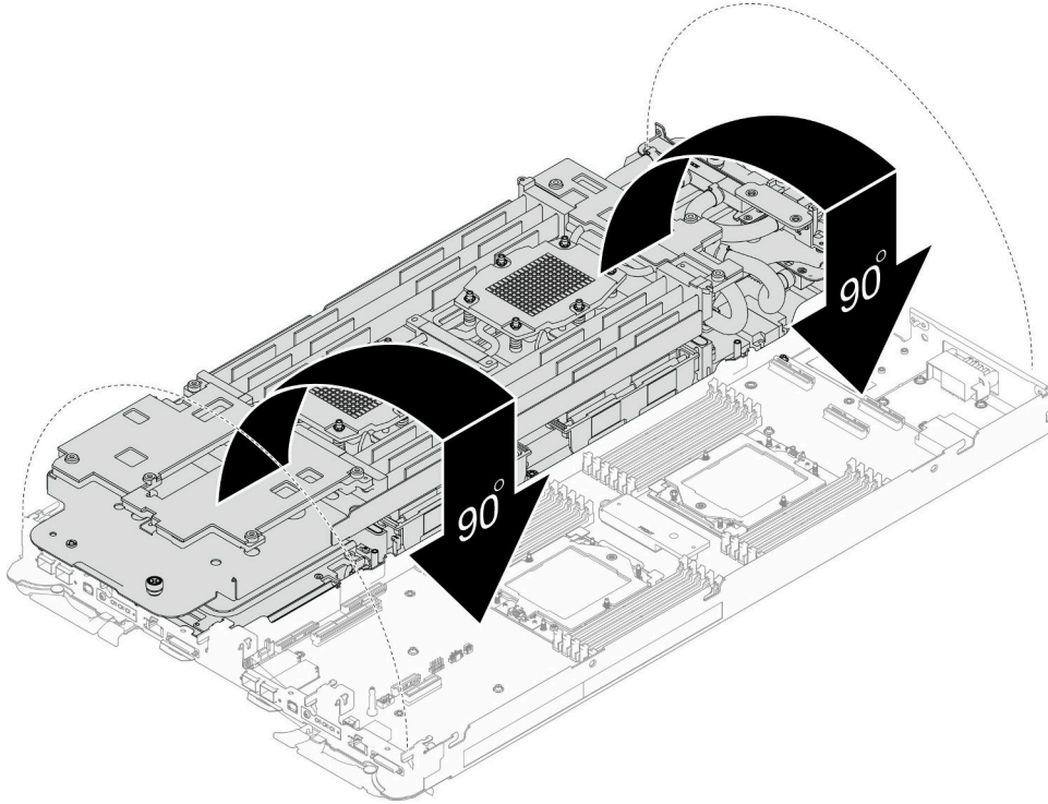
그림 210. 워터 루프 설치
