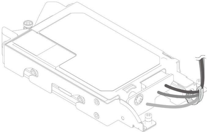
그림 112. 케이블 타이로 케이블 묶기
