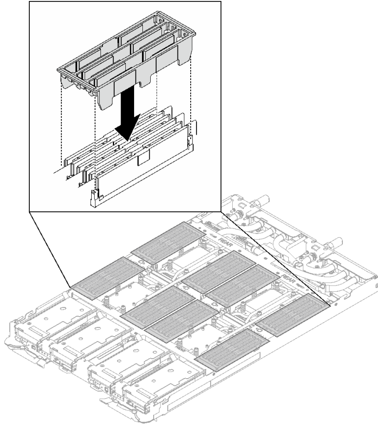
그림 134. DIMM 덮개 설치
