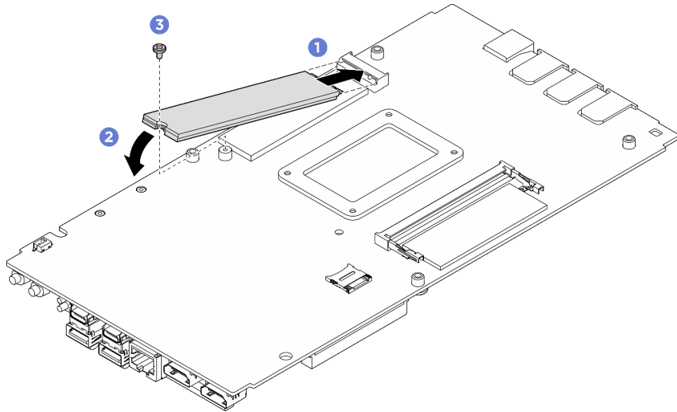
그림 110. M.2 드라이브 설치
