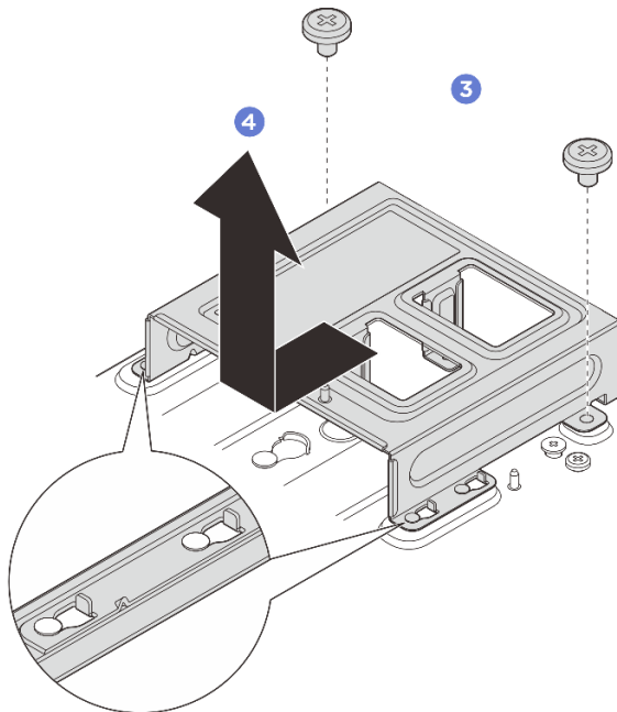
그림 63. 전원 어댑터 케이스 제거
