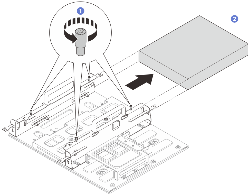
그림 21. 노드 슬리브에서 노드 제거
