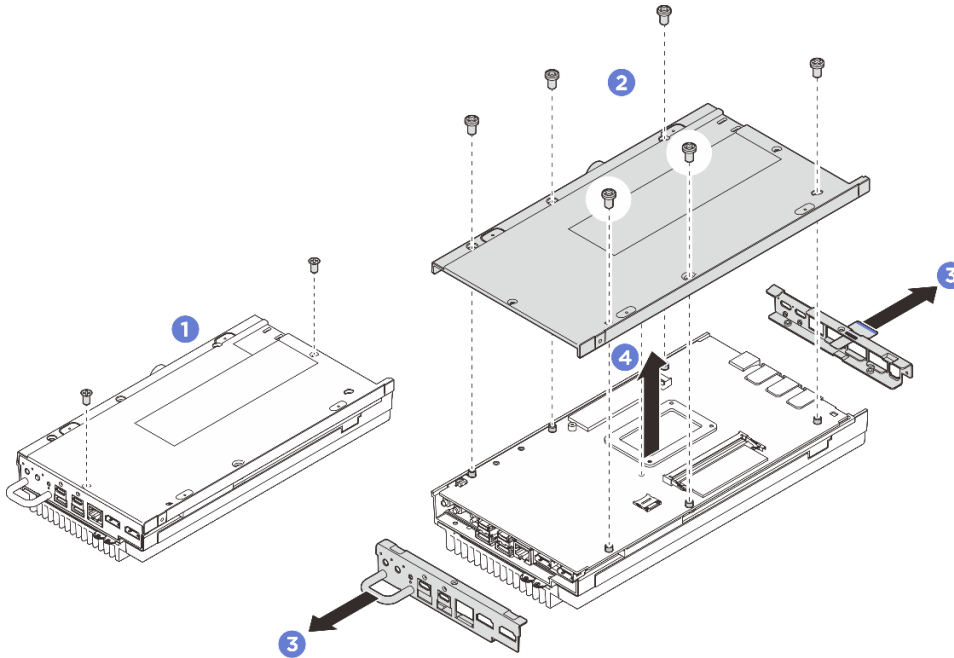
그림 132. 밀면 덮개 제거
