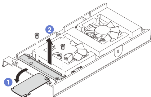
그림 81. 팬 브리지 케이블 덮개 제거
