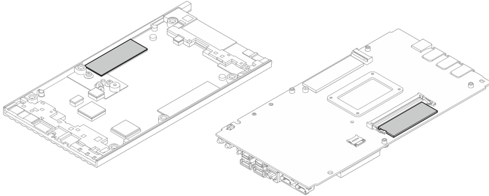
그림 120. 메모리 모듈 슬롯 2 열 패드(밀면 덮개 및 시스템 보드 측면)
