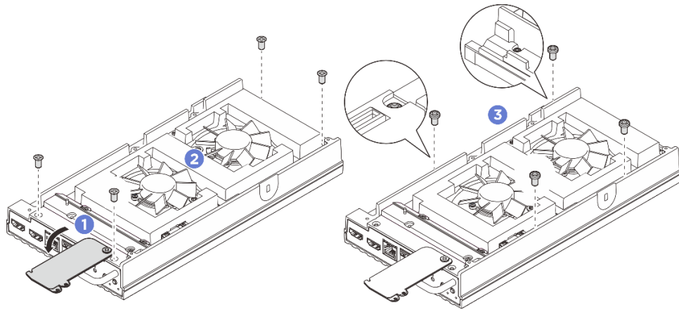
그림 124. 윗면 덮개에서 나사 제거
