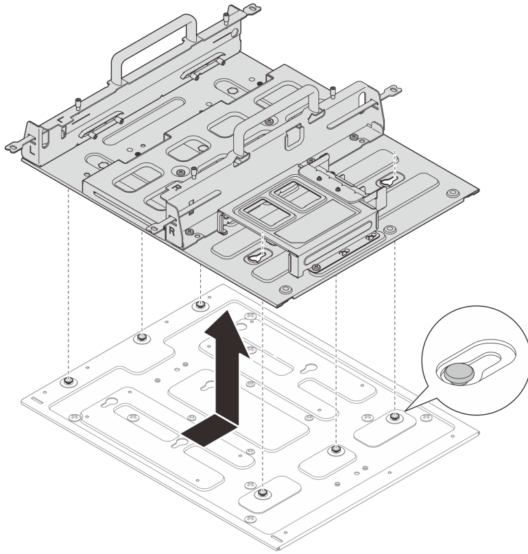
그림 47. 노드 슬리브 제거
