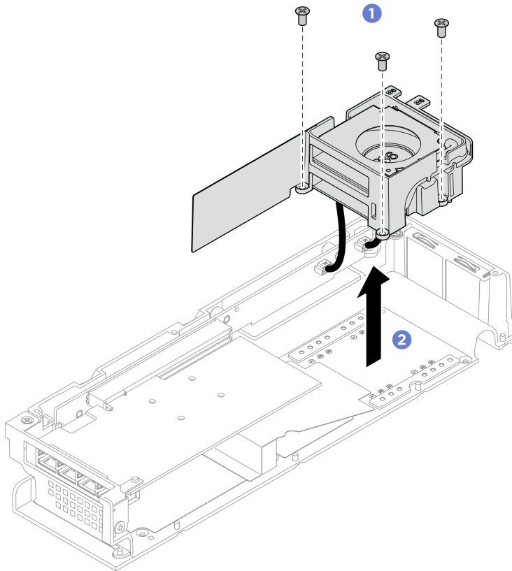
그림 166. 팬 모듈 제거
