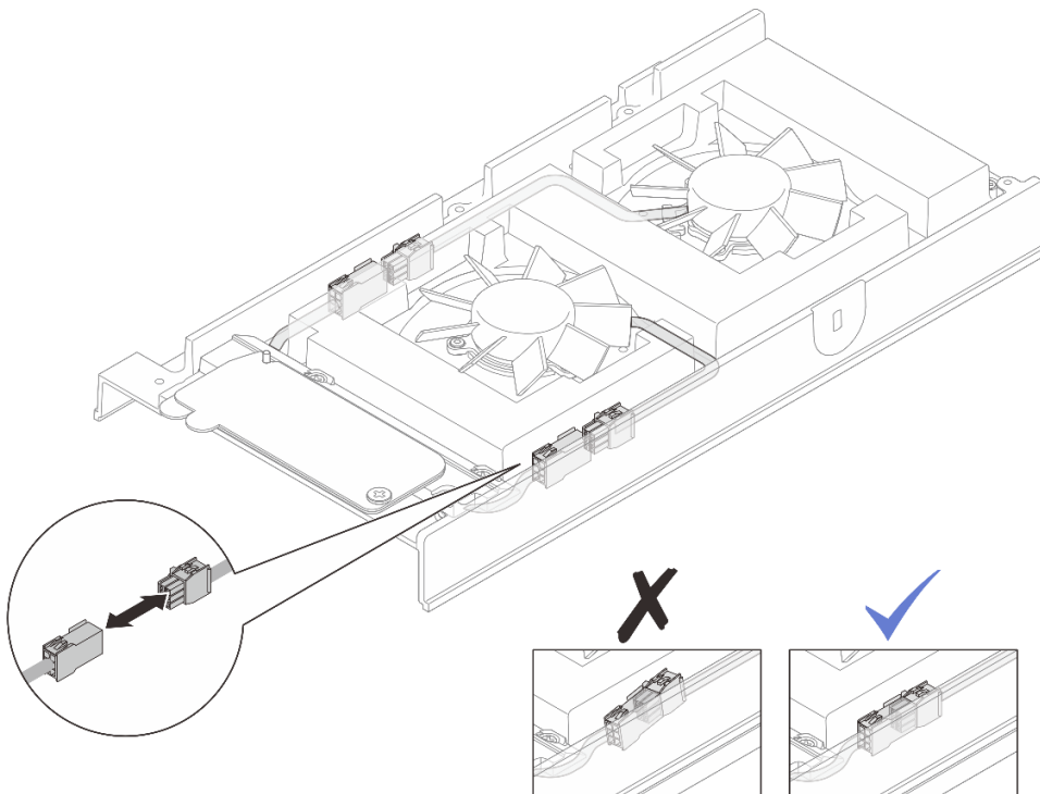
그림 88. 팬 브리지 케이블 재연결
