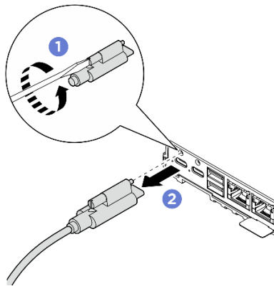
그림 69. 전원 케이블 제거
