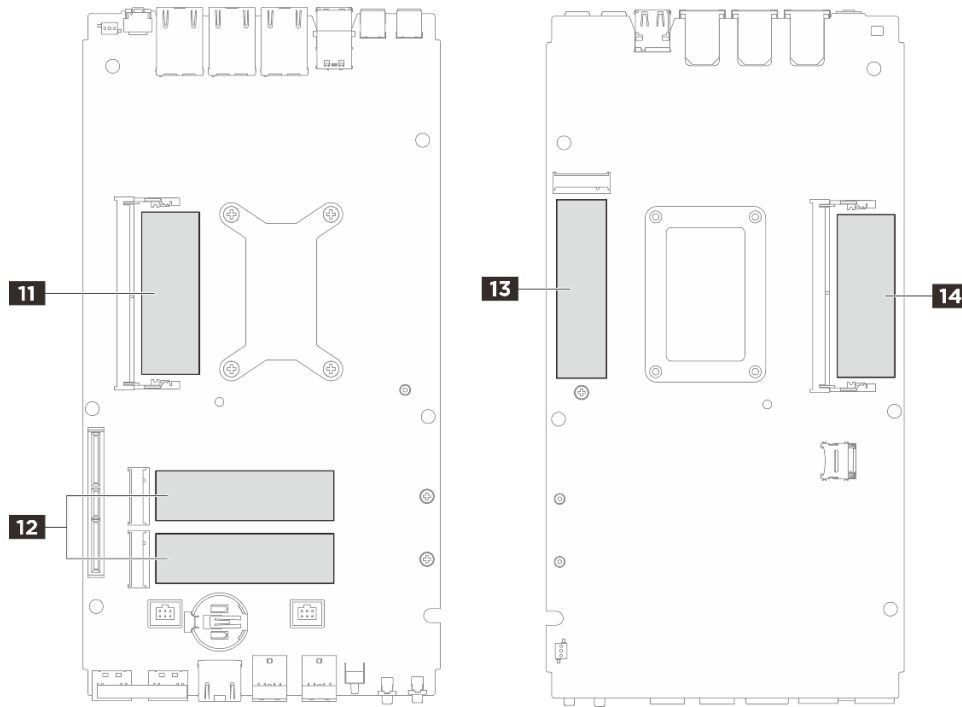
그림 4. 시스템 보드 - 열 패드 키트 식별 및 위치
