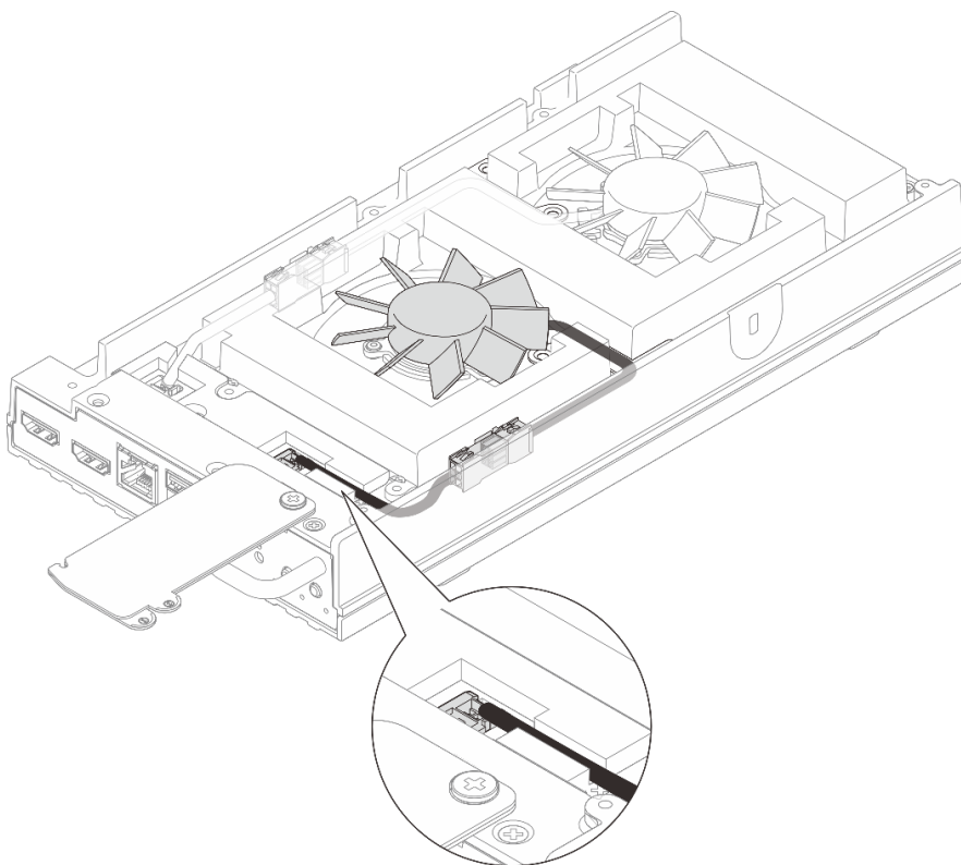
그림 86. 팬 커넥터 2의 케이블 배선
