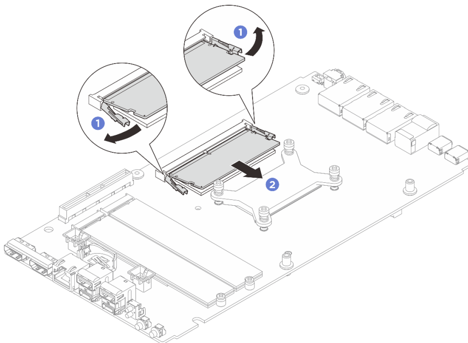
그림 117. 메모리 모듈 제거
