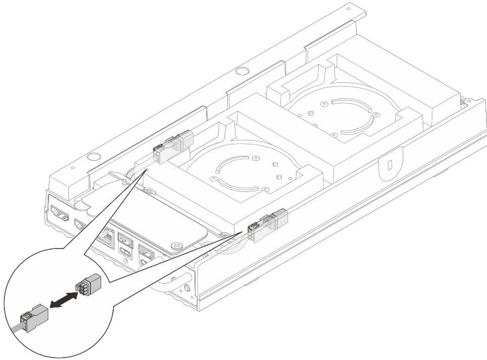
그림 91. 팬 브리지 케이블 먼지 필터 제거
