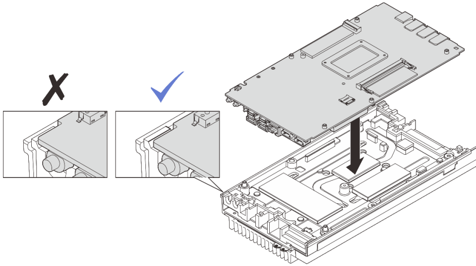
그림 154. 시스템 보드 설치
