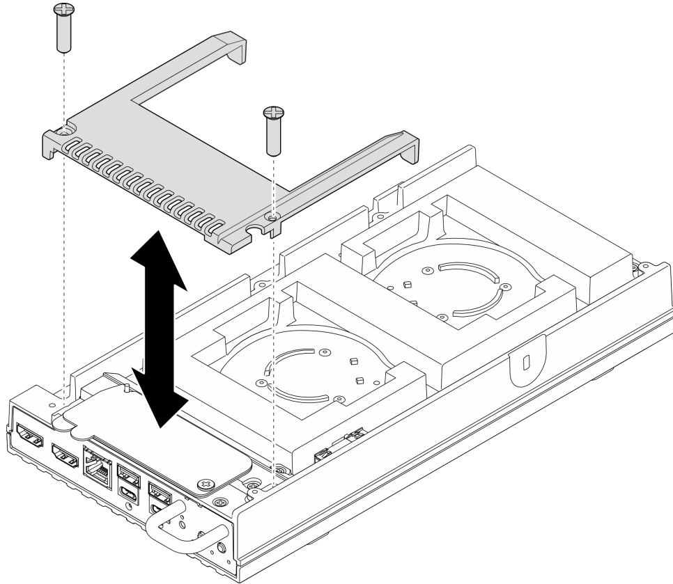
그림 90. 팬 슈라우드 제거
