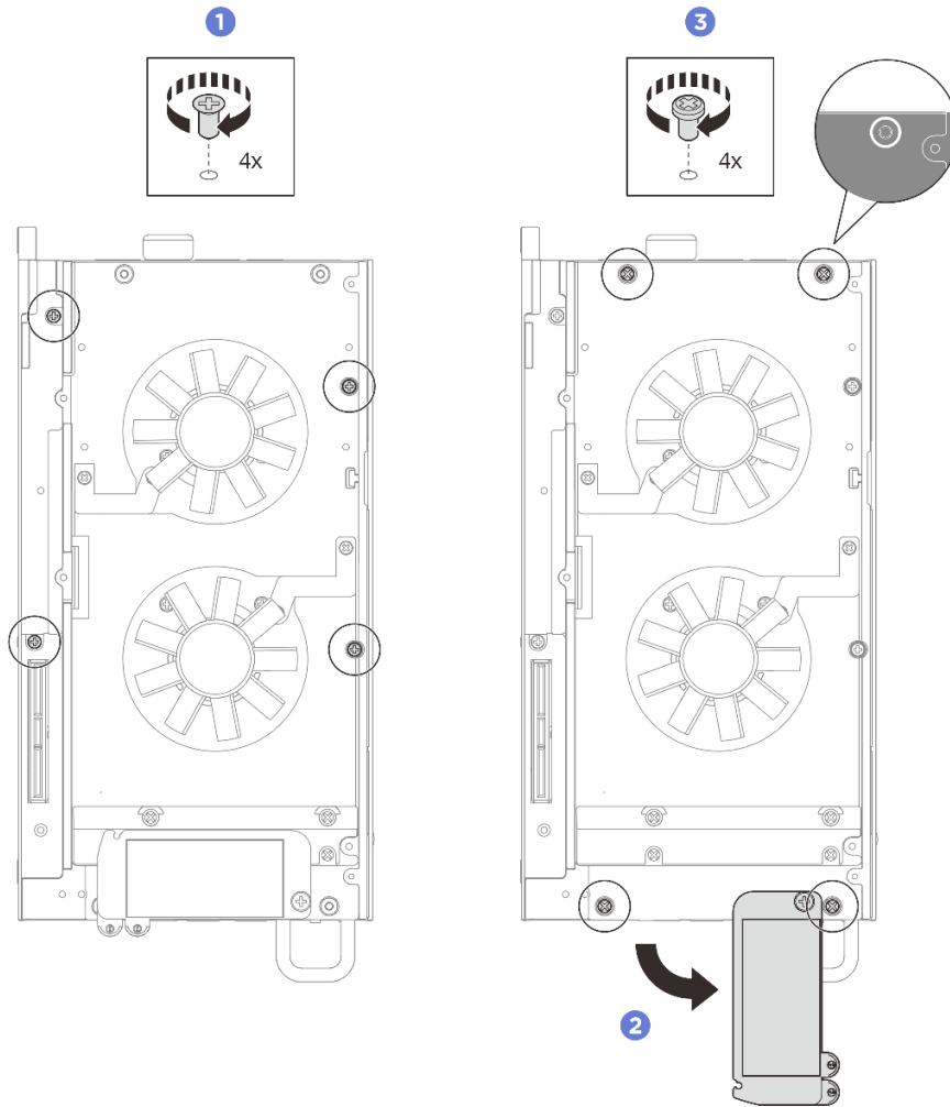
그림 147. 나사 설치
