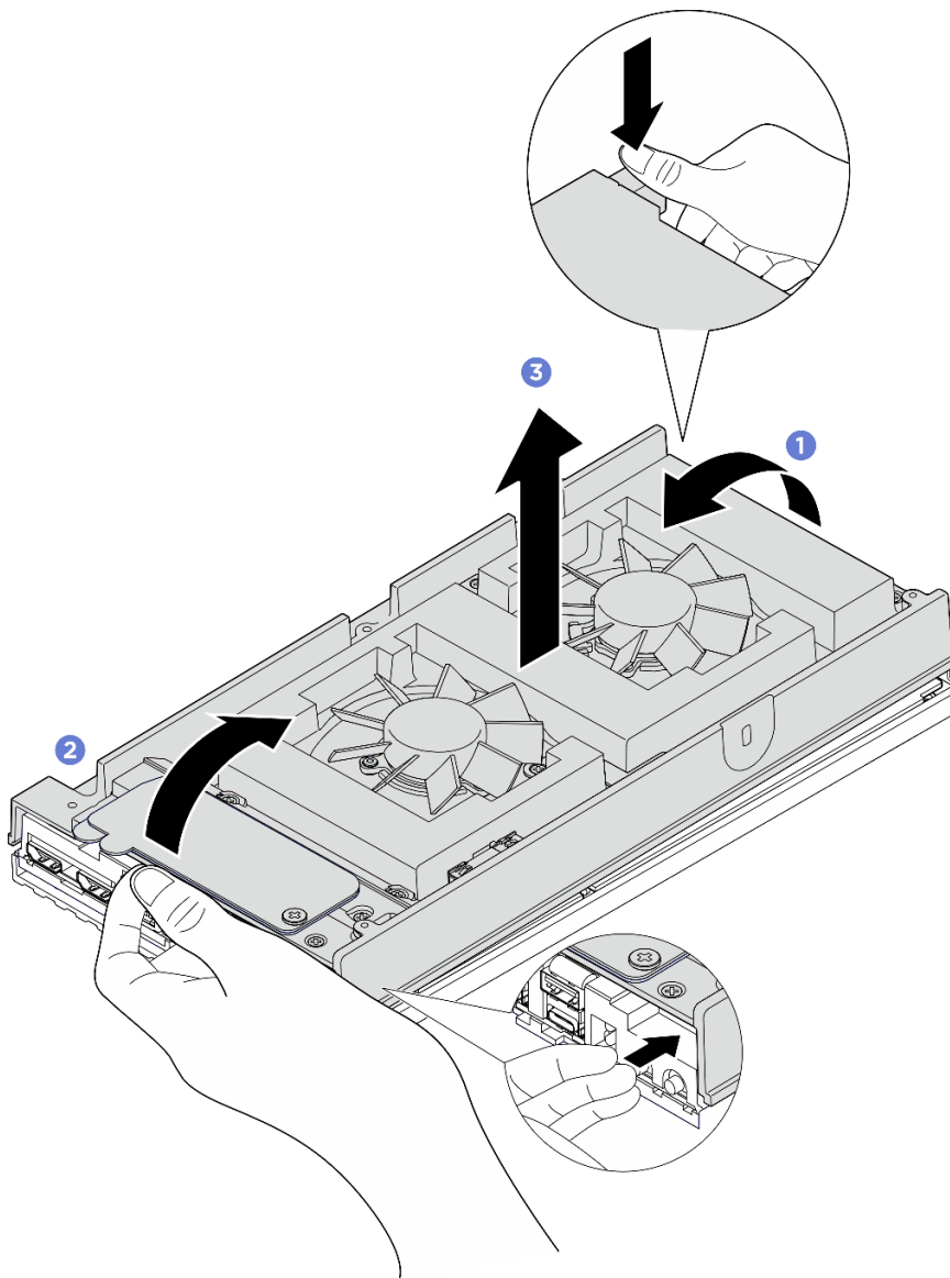
그림 126. 윗면 덮개 제거
