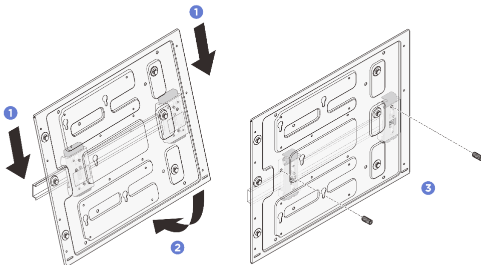
그림 49. DIN 레일 마운트 플레이트 설치
