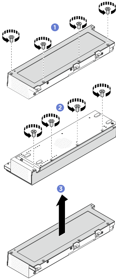
그림 164. 확장 윗면 덮개 제거
