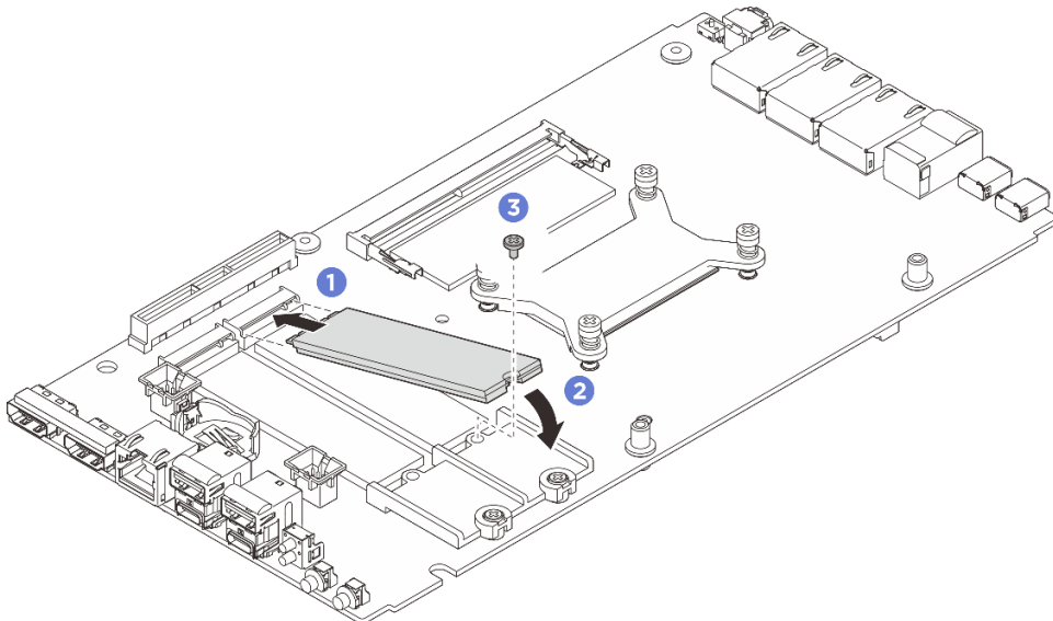
그림 115. M.2 드라이브 유형 2280 설치
