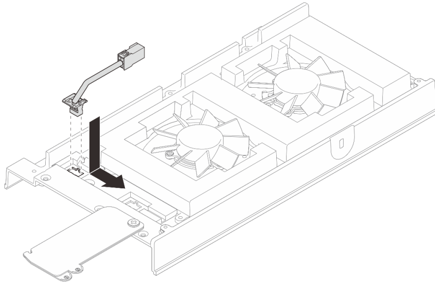
그림 84. 팬 브리지 케이블 설치
