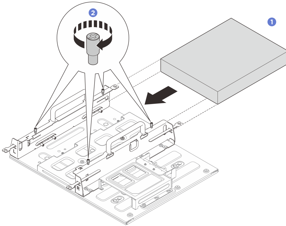
그림 53. 노드 슬리브에 노드 설치
