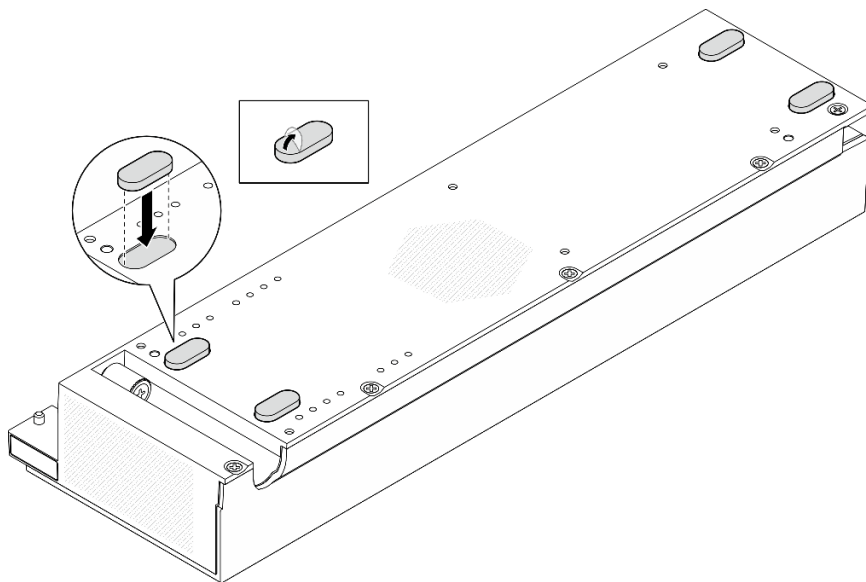
그림 57. PCIe 확장 키트에 고무 발 설치
