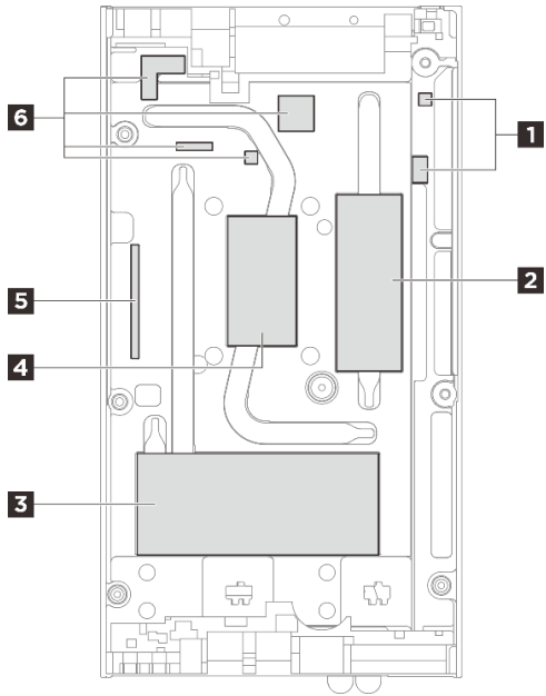
그림 2. 윗면 덮개 - 열 패드 키트 식별 및 위치
