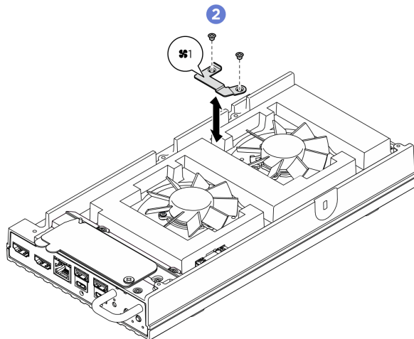
그림 101. 팬 1 브래킷의 나사 위치
