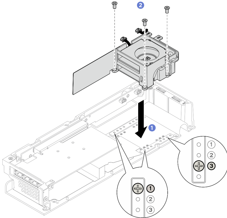
그림 167. 팬 모듈 설치
