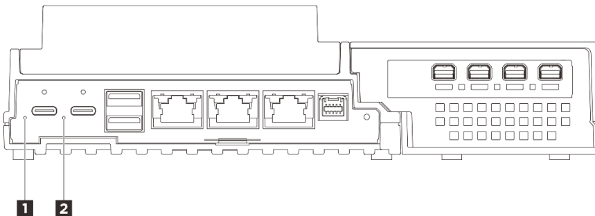
그림 184. 뒷면 LED
