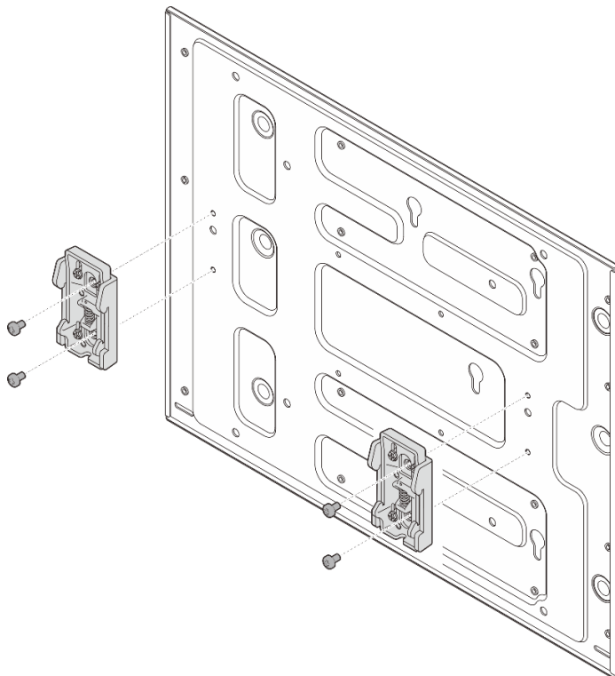
그림 44. DIN 레일 클립 제거
