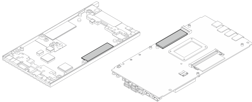
그림 109. M.2 드라이브 슬롯 1 열 패드(밀면 덮개 및 시스템 보드 측면)
