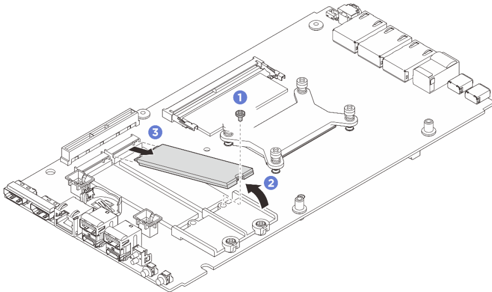
그림 107. M.2 드라이브(2280 폼 팩터) 제거
