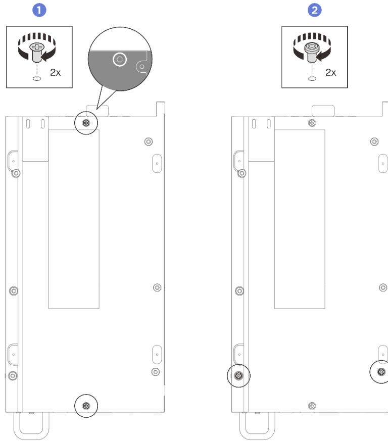
그림 130. 나사 설치
