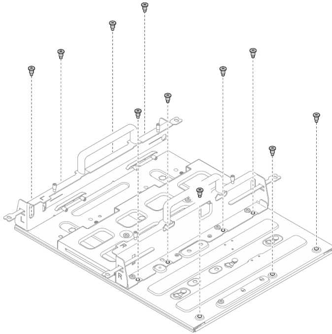
그림 36. 확장 키트를 사용해 노드 슬리브 설치
