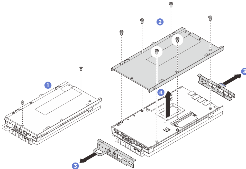
그림 137. 밑면 덮개 제거
