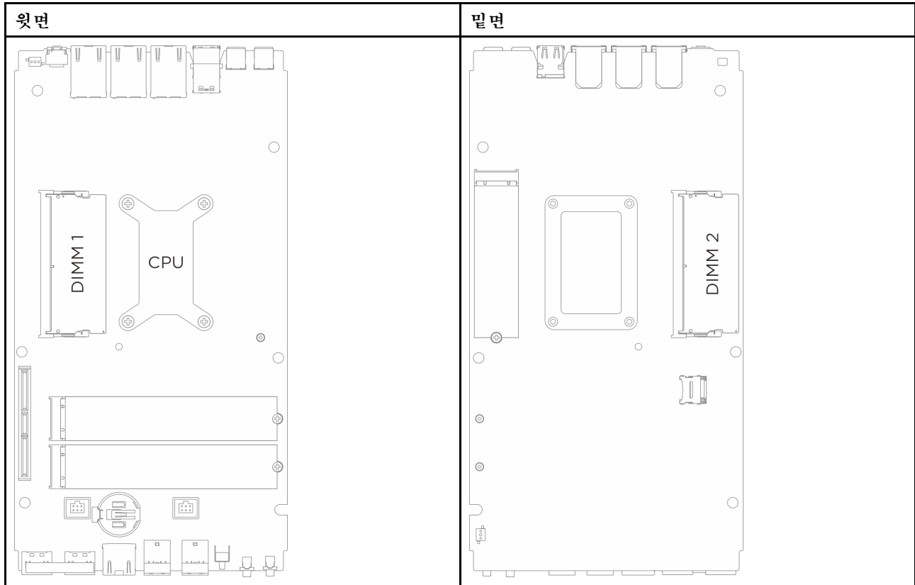
그림 1. 메모리 모듈 및 프로세서 레이아웃
