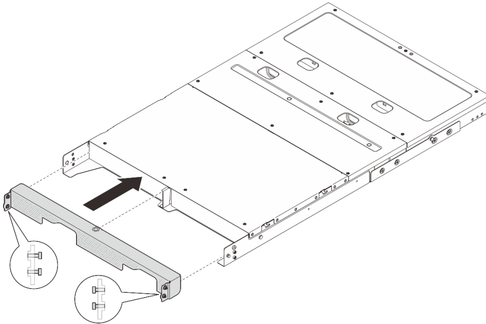
그림 19. 운반 브래킷 설치
