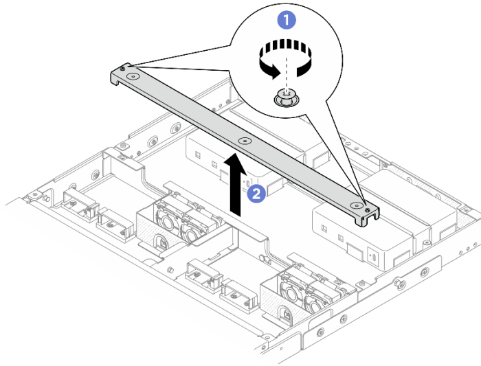
그림 68. 크로스바 제거
