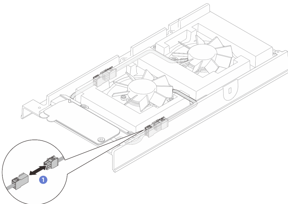
그림 82. 팬 브리지 케이블 분리
