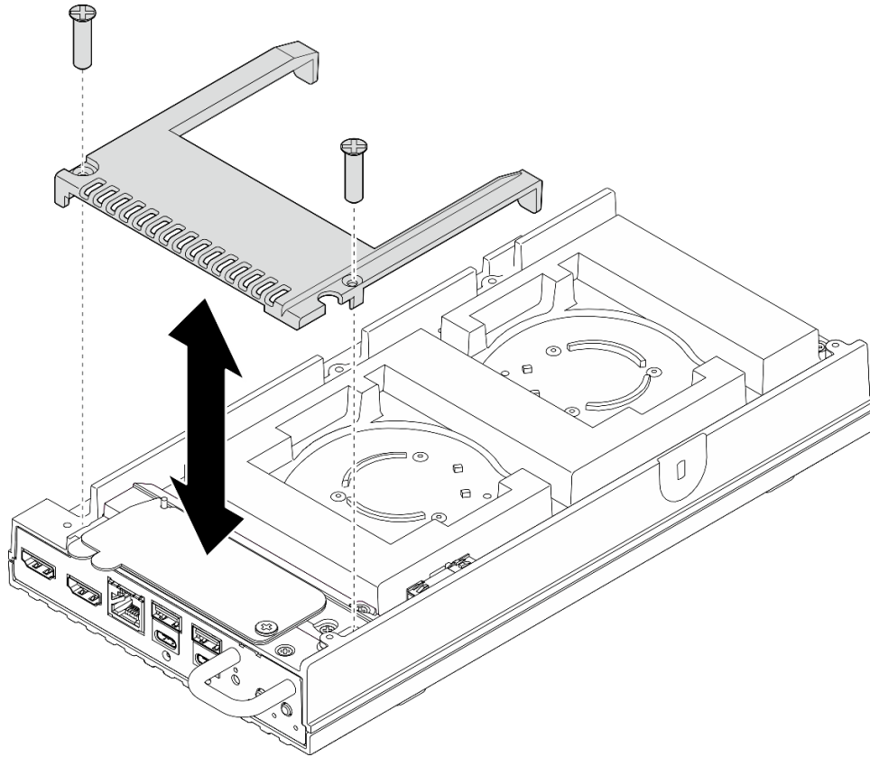
그림 95. 팬 슈라우드 설치
