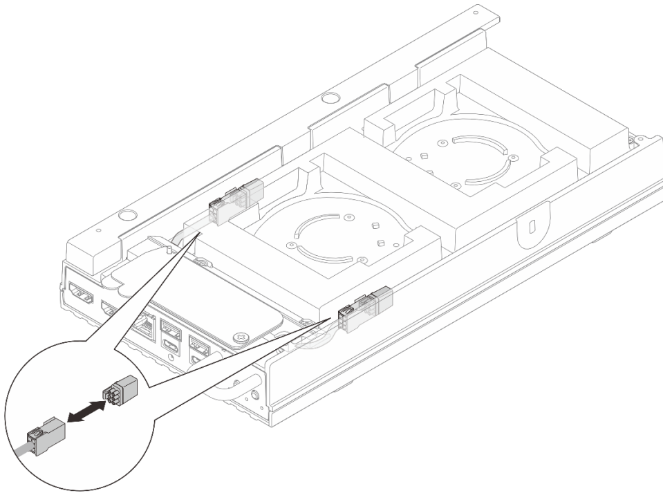
그림 94. 팬 브리지 케이블 먼지 필터 설치
