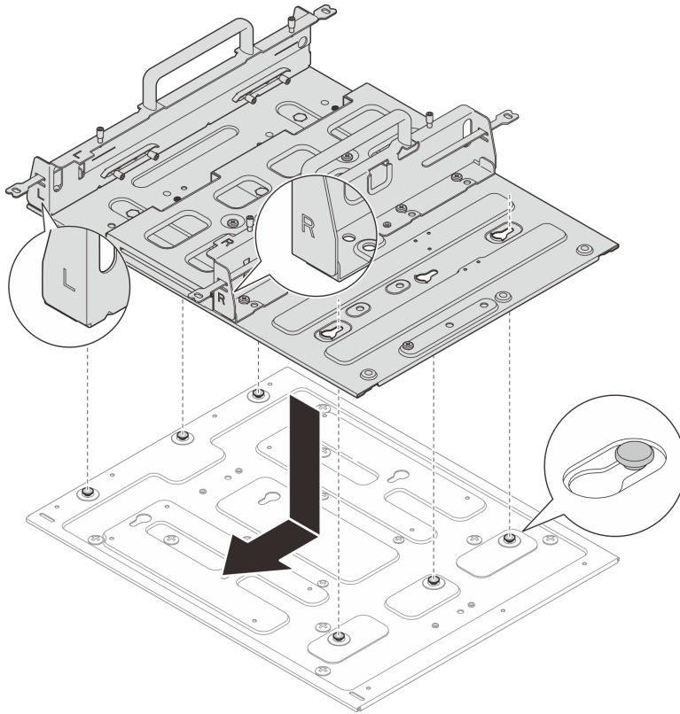
그림 50. 노드 슬리브 설치
