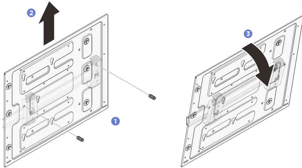
그림 43. DIN 레일 마운트 플레이트 제거
