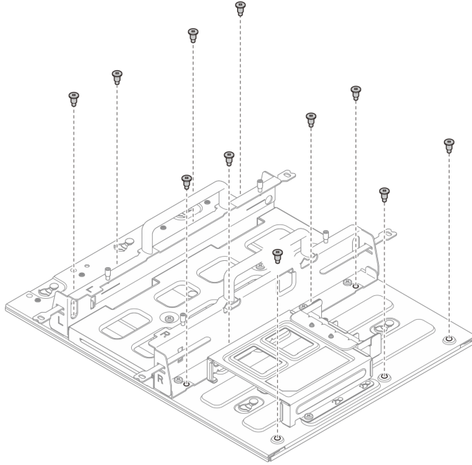
그림 46. 확장 키트를 사용하지 않고 노드 슬리브 제거
