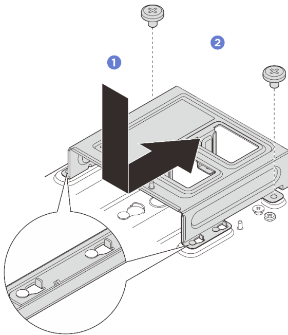
그림 64. 전원 어댑터 브래킷 설치
