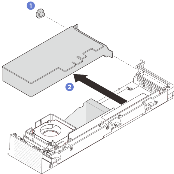
그림 177. PCIe 어댑터 제거
