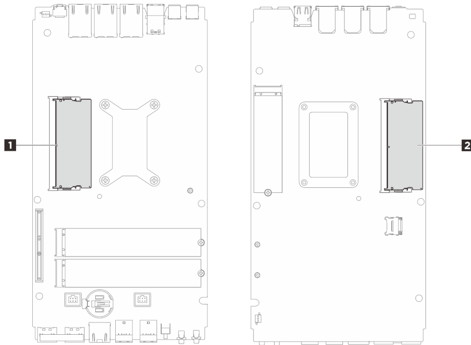
그림 116. 메모리 모듈 및 프로세서 레이아웃
