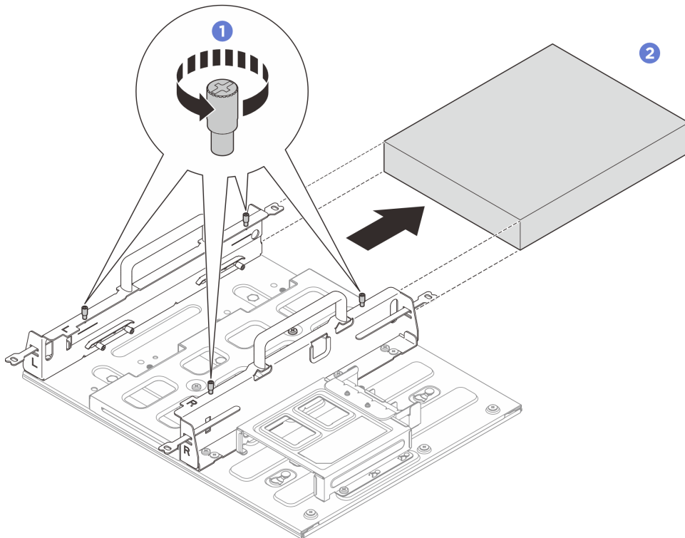
그림 39. 노드 슬리브에서 노드 제거
