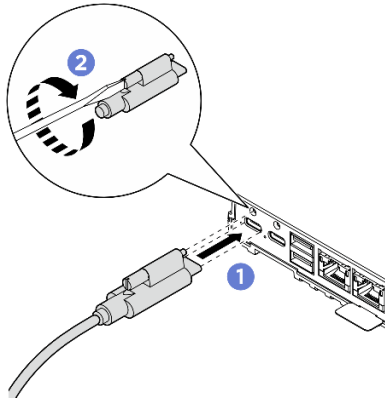
그림 72. 전원 케이블 설치
