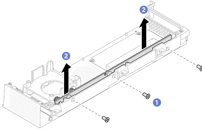
그림 175. PCIe 라이저 카드 제거
