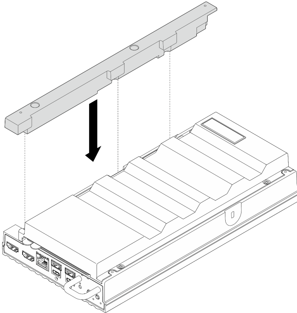
그림 79. 확장 필러 설치
