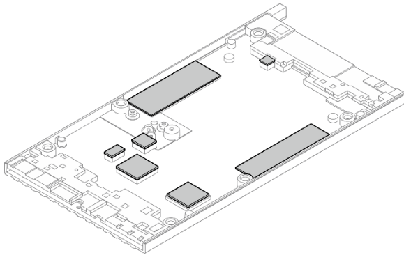
그림 152. 밑면 덮개 열 패드
