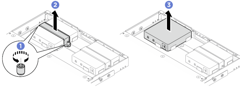
그림 70. 전원 어댑터 제거
