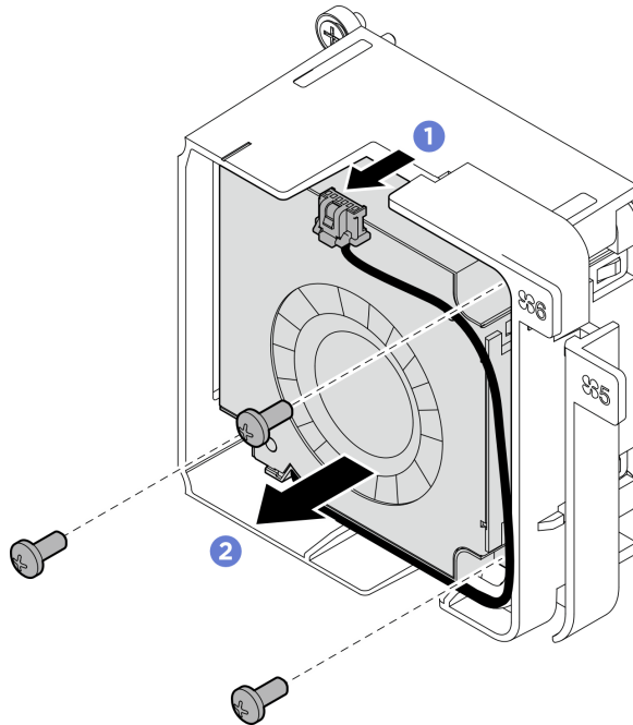
그림 169. 팬 6 제거
