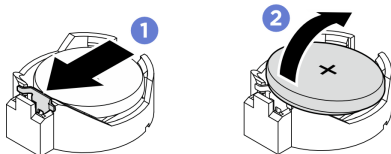
그림 75. CMOS 배터리 제거
