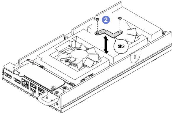
그림 98. 팬 2 브래킷의 나사 위치
