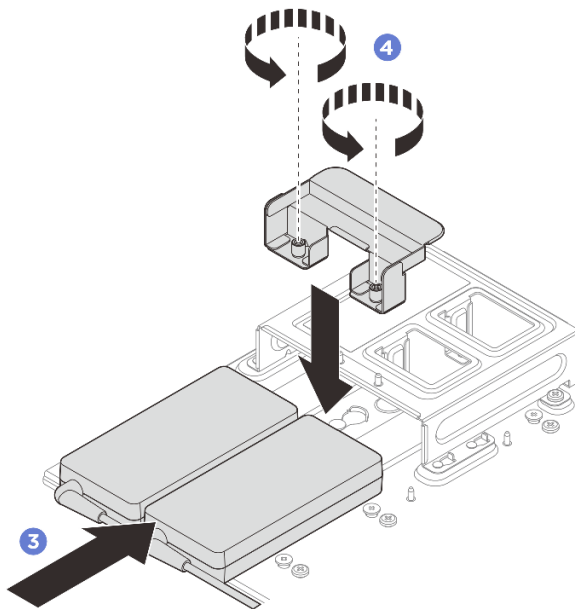
그림 66. 전원 어댑터 설치
