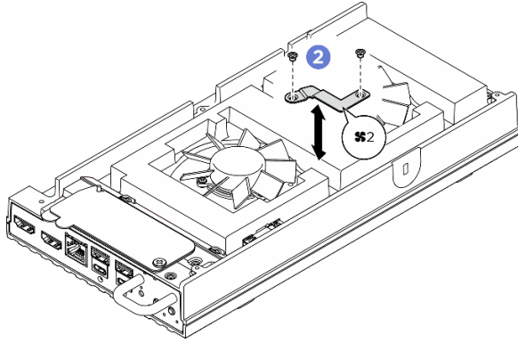
그림 102. 팬 2 브래킷의 나사 위치
