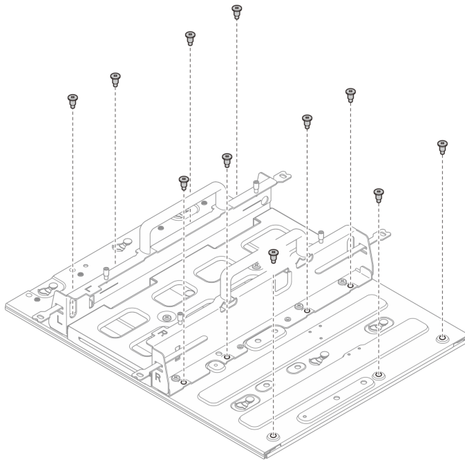
그림 52. 확장 키트를 사용하지 않고 노드 슬리브 설치
