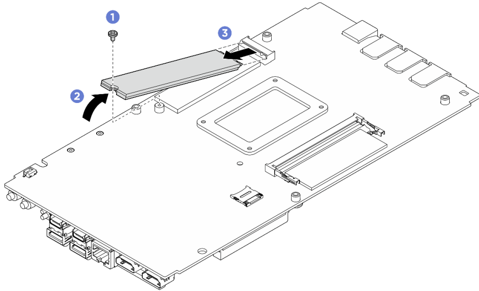
그림 105. M.2 드라이브 제거
