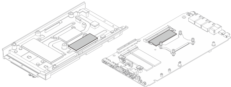
그림 119. 메모리 모듈 슬롯 1 열 패드(윗면 덮개 및 시스템 보드 측면)
