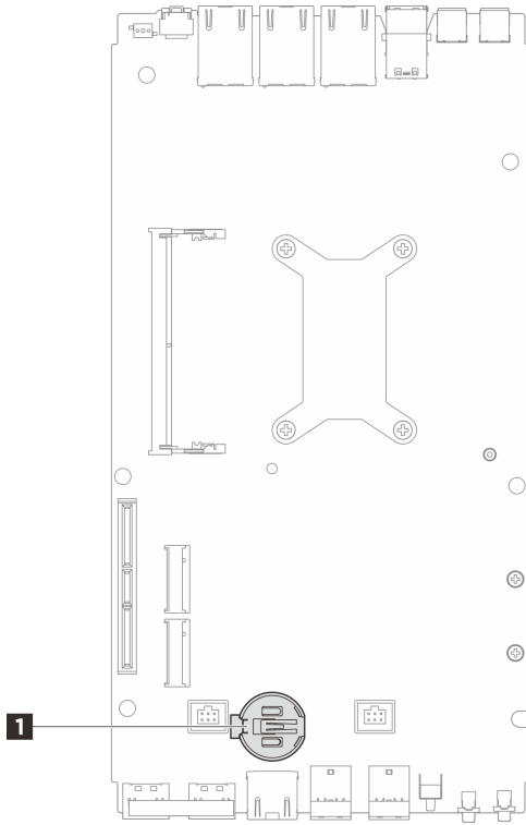
그림 74. CMOS 배터리 위치
