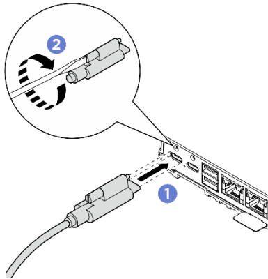
그림 59. 전원 케이블 설치
