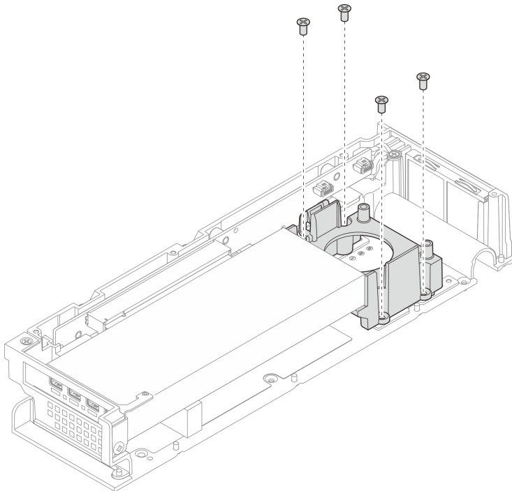
그림 174. 지지 조절 장치 설치
