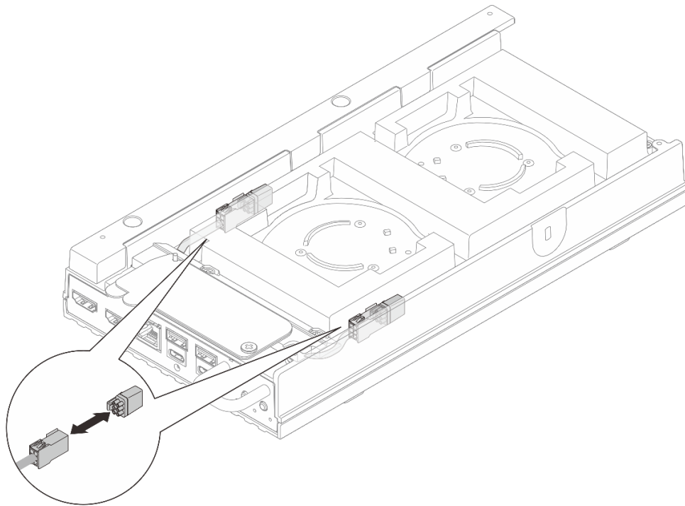
그림 92. 팬 브리지 케이블 먼지 필터 제거
