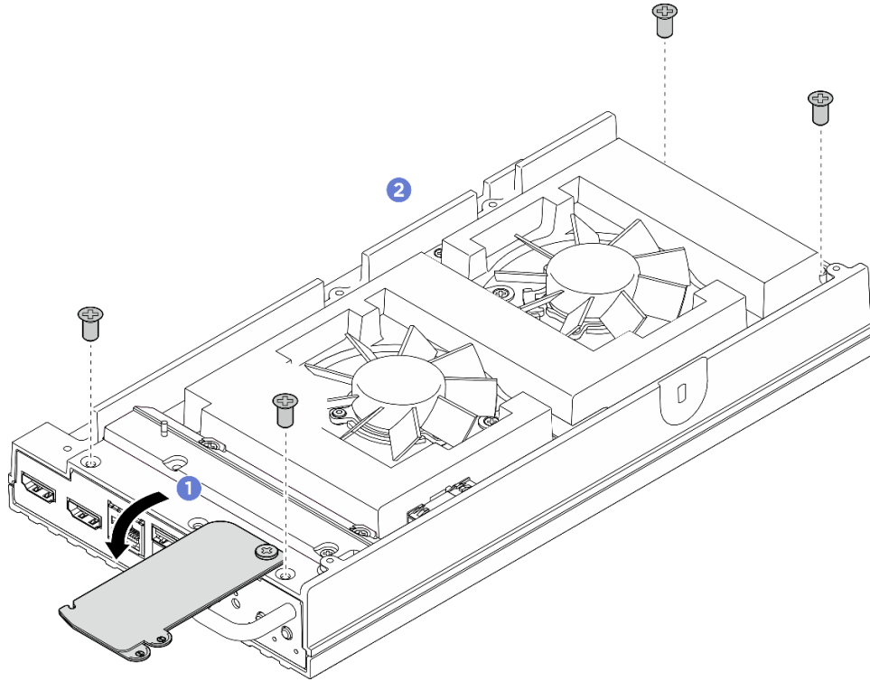
그림 131. 뒷면 덮개에서 나사 제거
