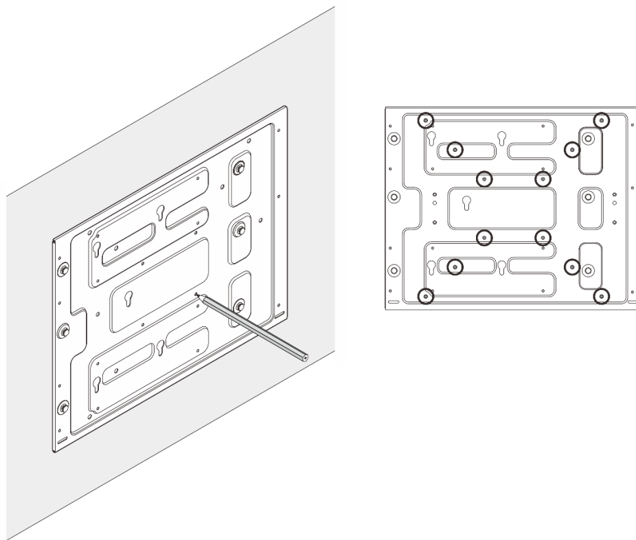
그림 31. 나사 구멍 위치
