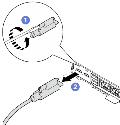
그림 60. 전원 케이블 제거
