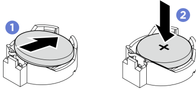
그림 77. CMOS 배터리 설치
