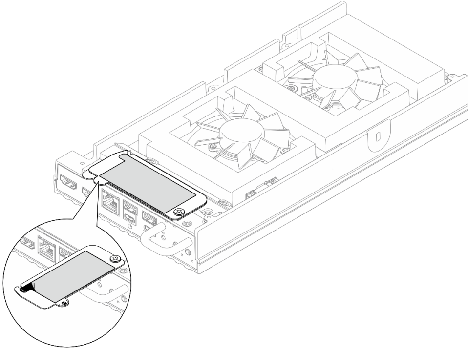
그림 153. 탈착식 정보 탭에 있는 Lenovo XClarity Controller 네트워크 액세스 레이블
