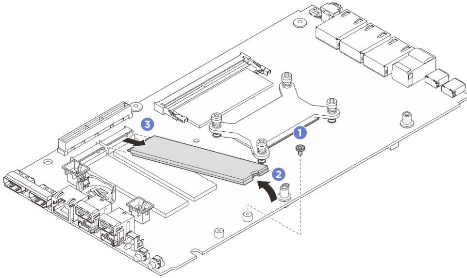
그림 106. M.2 드라이브 제거(22110 폼 팩터)
