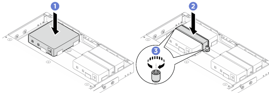
그림 71. 전원 어댑터 설치
