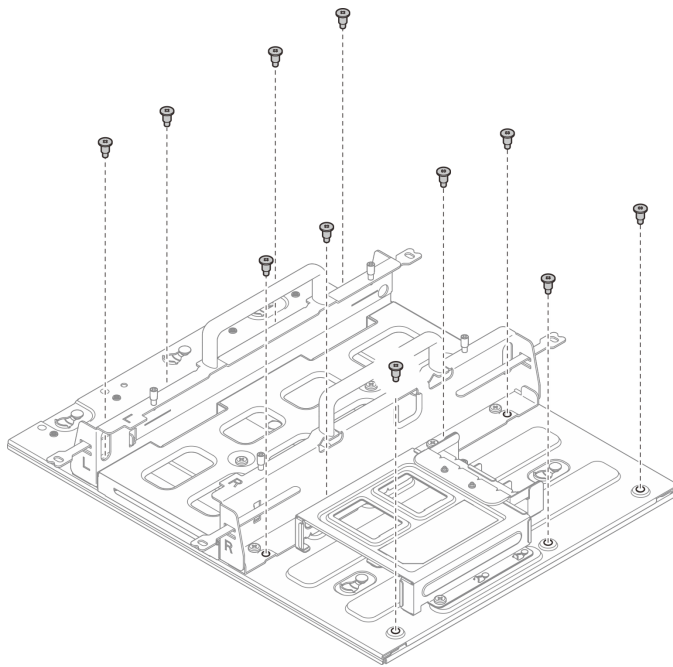
그림 41. 확장 키트를 사용하지 않고 노드 슬리브 제거
