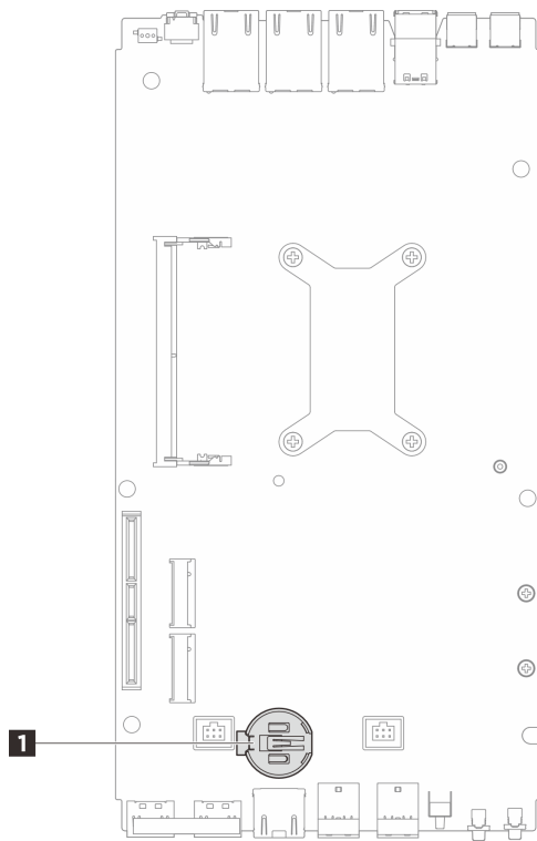
그림 76. CMOS 배터리 위치
