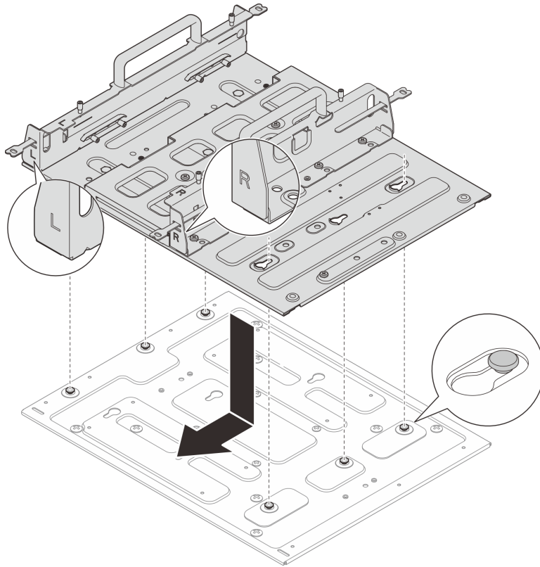
그림 35. 노드 슬리브 설치
