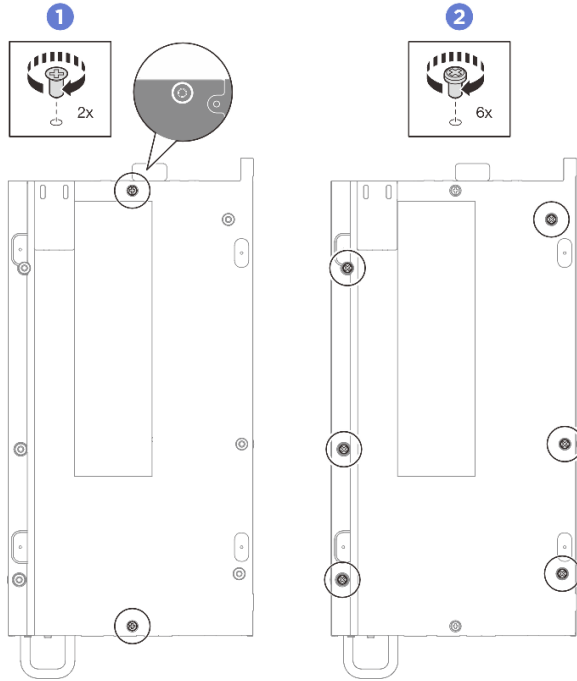
그림 156. 나사 설치
