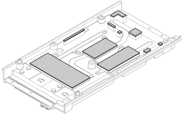
그림 140. 윗면 덮개 열 패드
