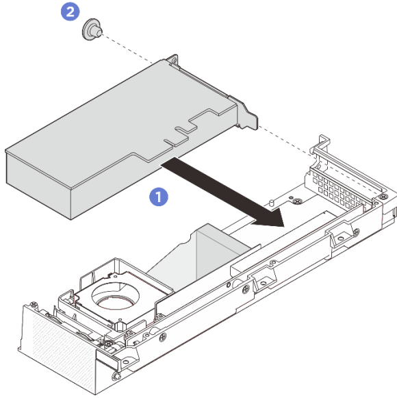
그림 178. PCIe 어댑터 설치
