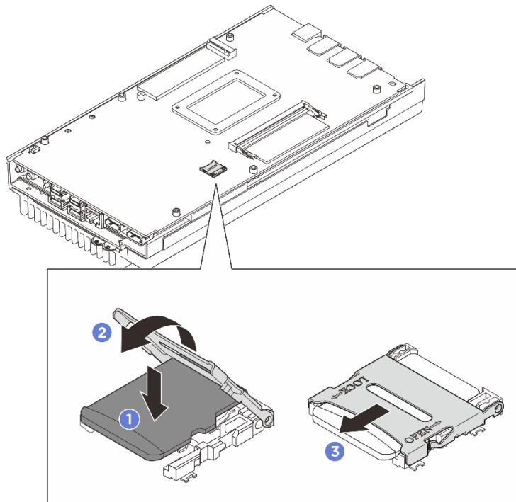
그림 123. MicroSD 카드 설치
