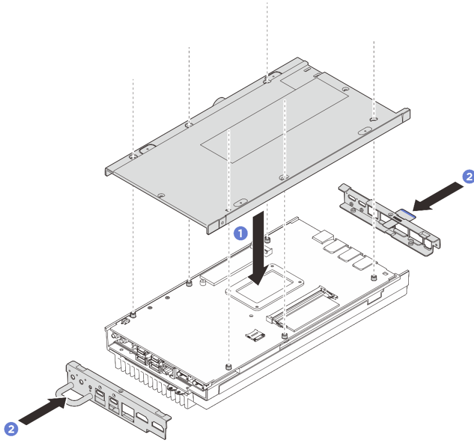
그림 134. 밀면 덮개 설치
