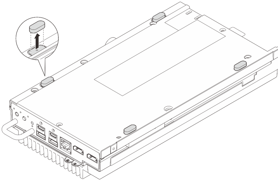
그림 54. 노드에서 고무 발 제거
