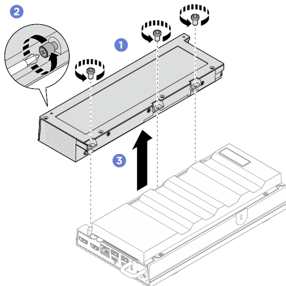
그림 162. 확장 키트 제거
