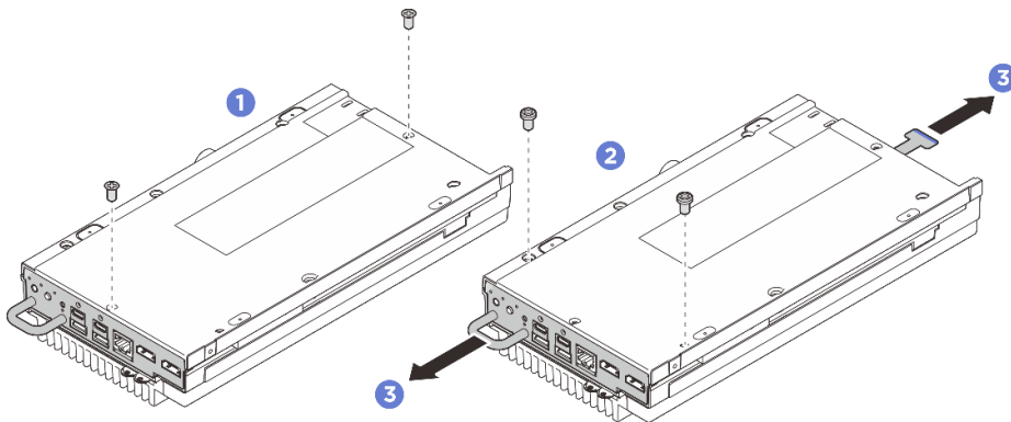
그림 125. 앞면 및 뒷면 I/O 브래킷 제거
