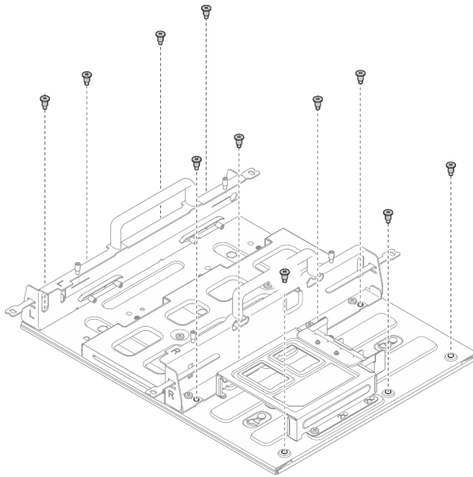
그림 40. 확장 키트를 사용해 노드 슬리브 제거
