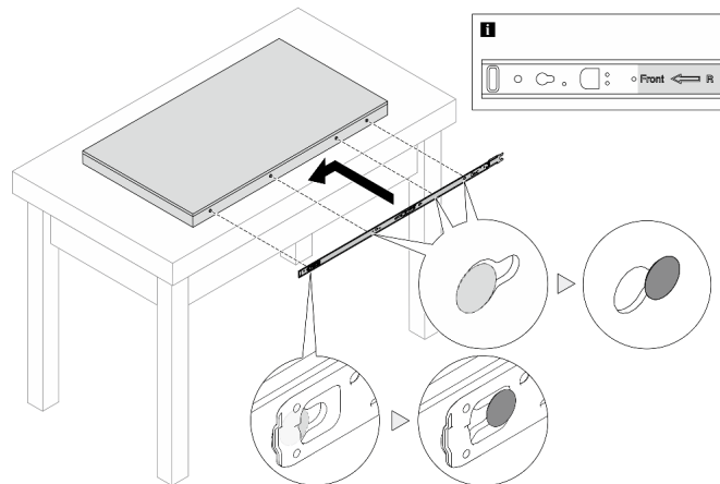
그림 10. 서버에 내부 레일 설치
