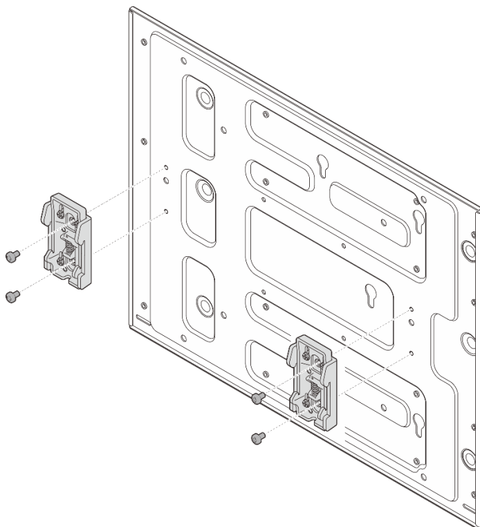
그림 48. DIN 레일 클립 설치
