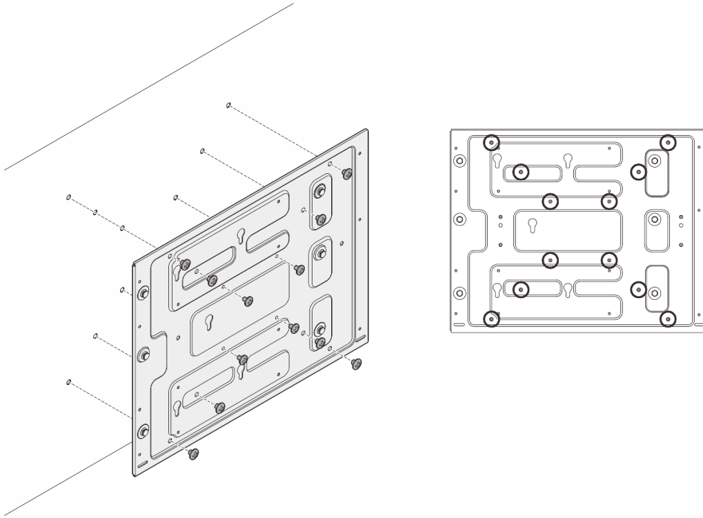
그림 25. 벽 마운트 플레이트 제거
