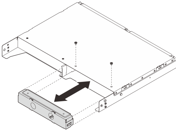
그림 16. 노드 필터 제거
