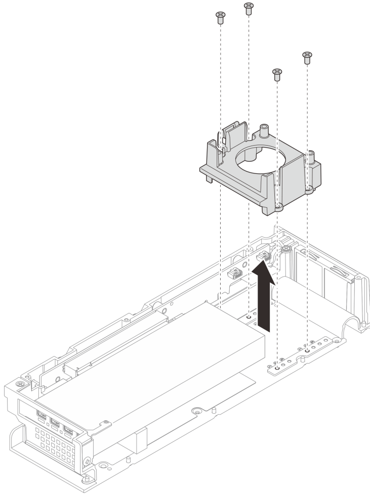
그림 172. 지지 조절 장치 제거
