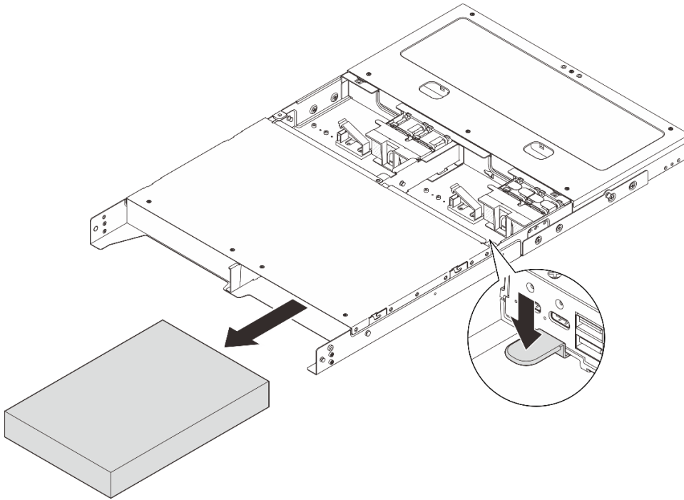
그림 7. 노드 제거
