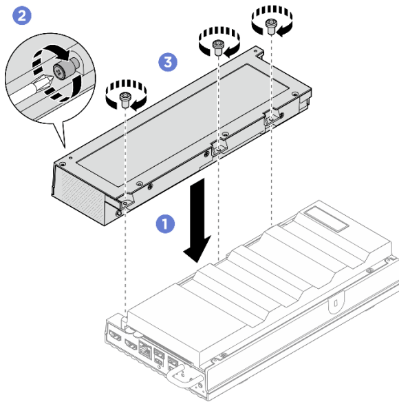
그림 163. 확장 키트 설치
