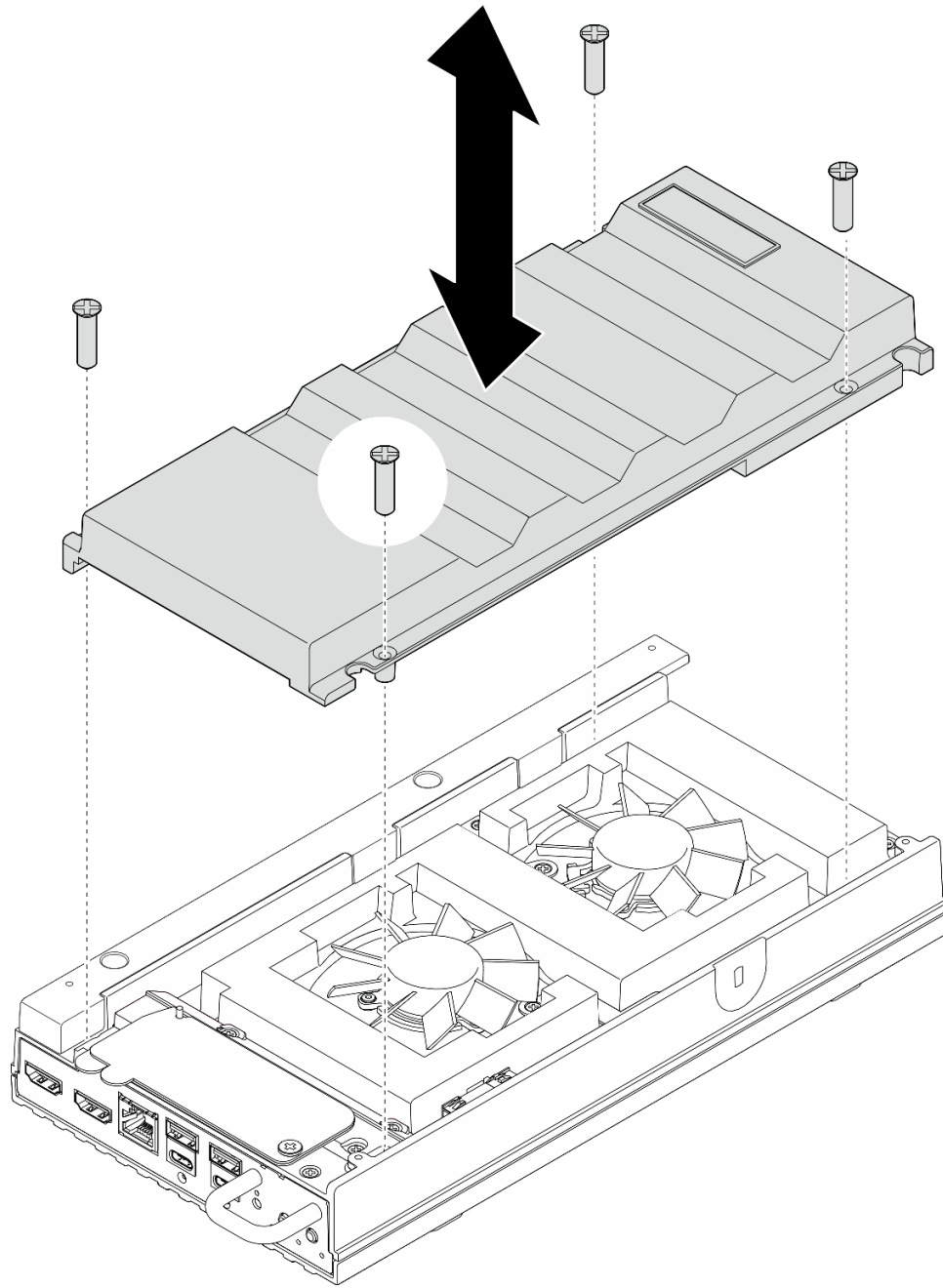
그림 89. 팬 슈라우드 제거
