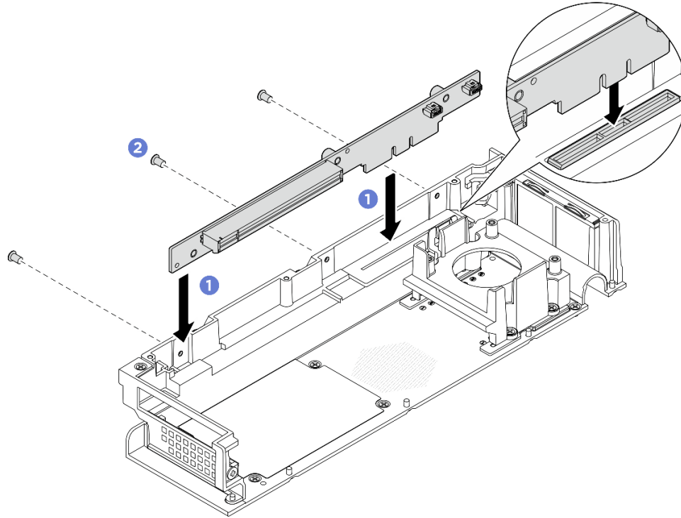
그림 176. PCIe 라이저 카드 설치
