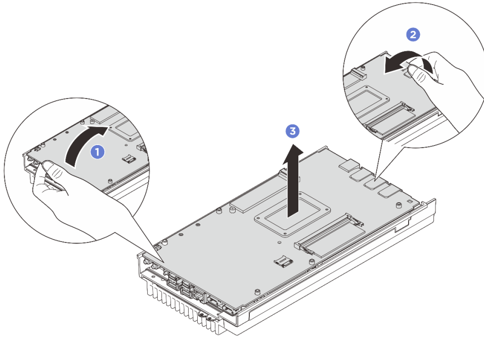
그림 138. 시스템 보드 분해
