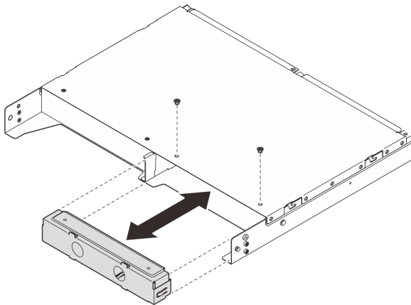
그림 8. 노드 필터 설치
