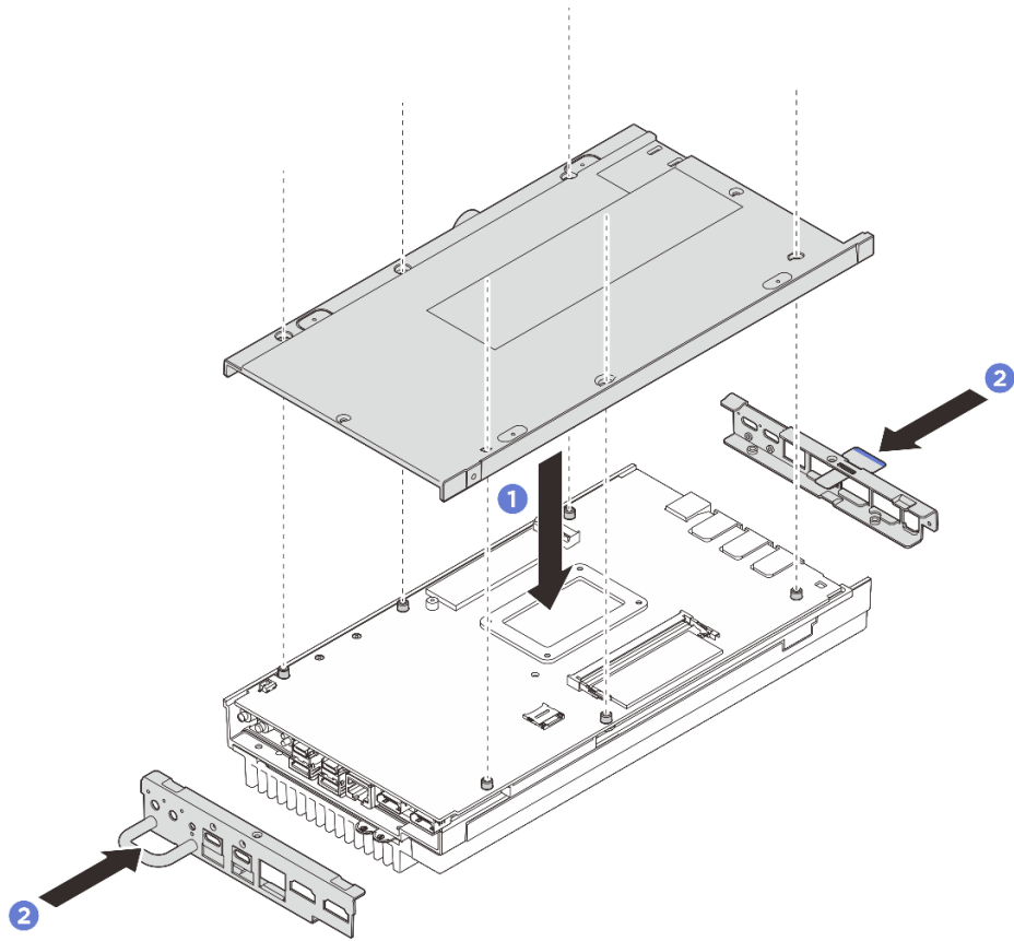
그림 145. 밀면 덮개 설치
