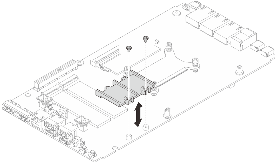
그림 114. M.2 홀더 설치
