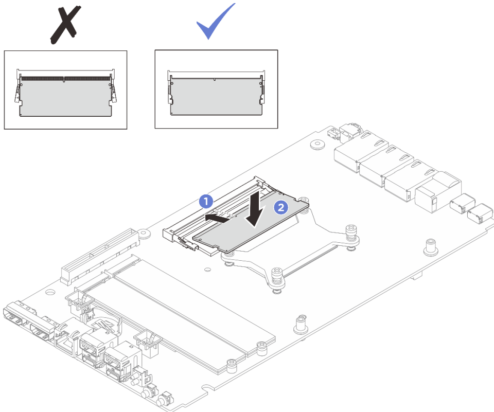
그림 121. 메모리 모듈 설치
