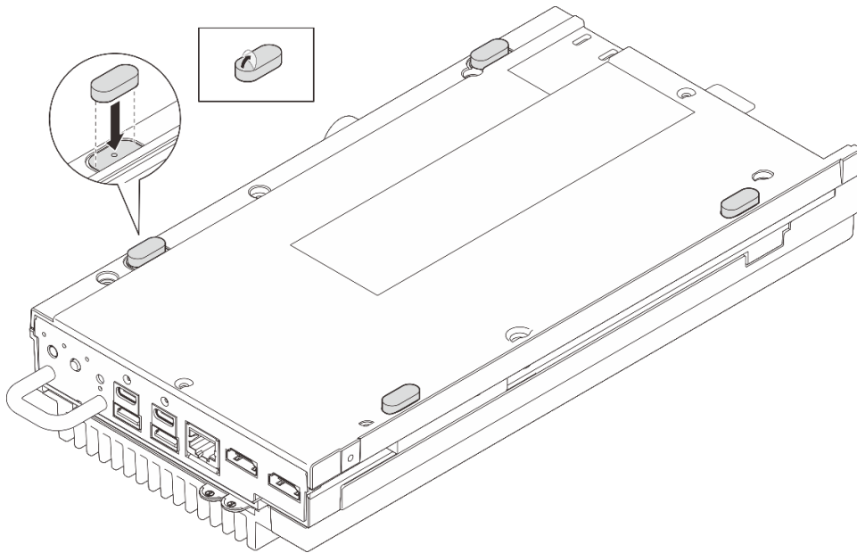
그림 56. 노드에 고무 발 설치
