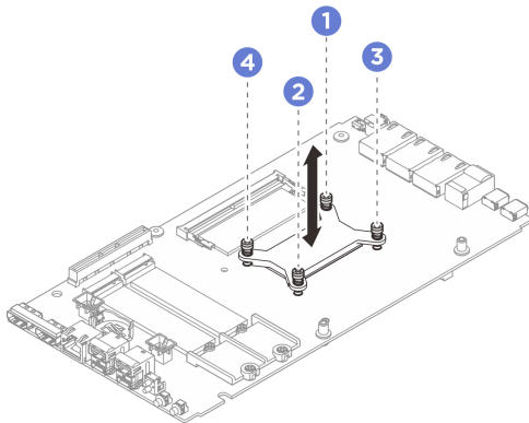
그림 143. 프로세서 방열판 설치
