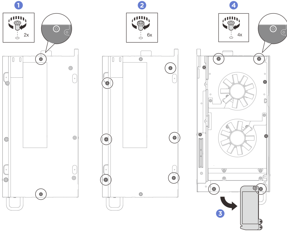
그림 135. 모든 나사 조이기
