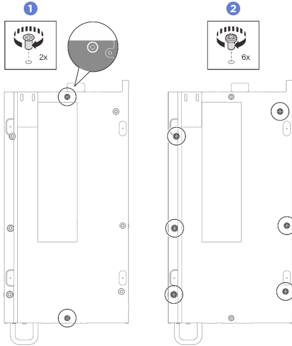
그림 146. 나사 설치
