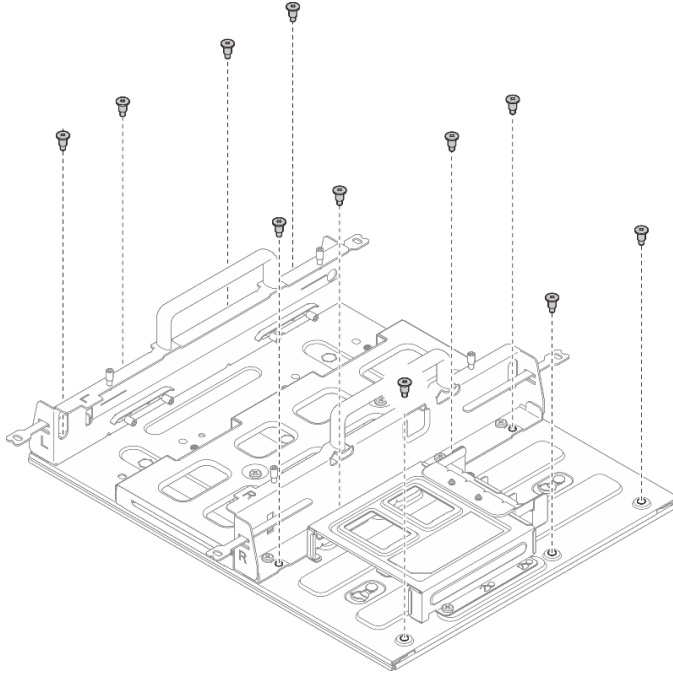
그림 22. 확장 키트를 사용해 노드 슬리브 제거
