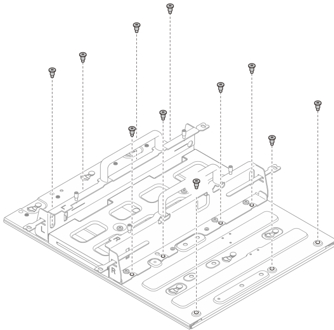
그림 37. 확장 키트를 사용하지 않고 노드 슬리브 설치
