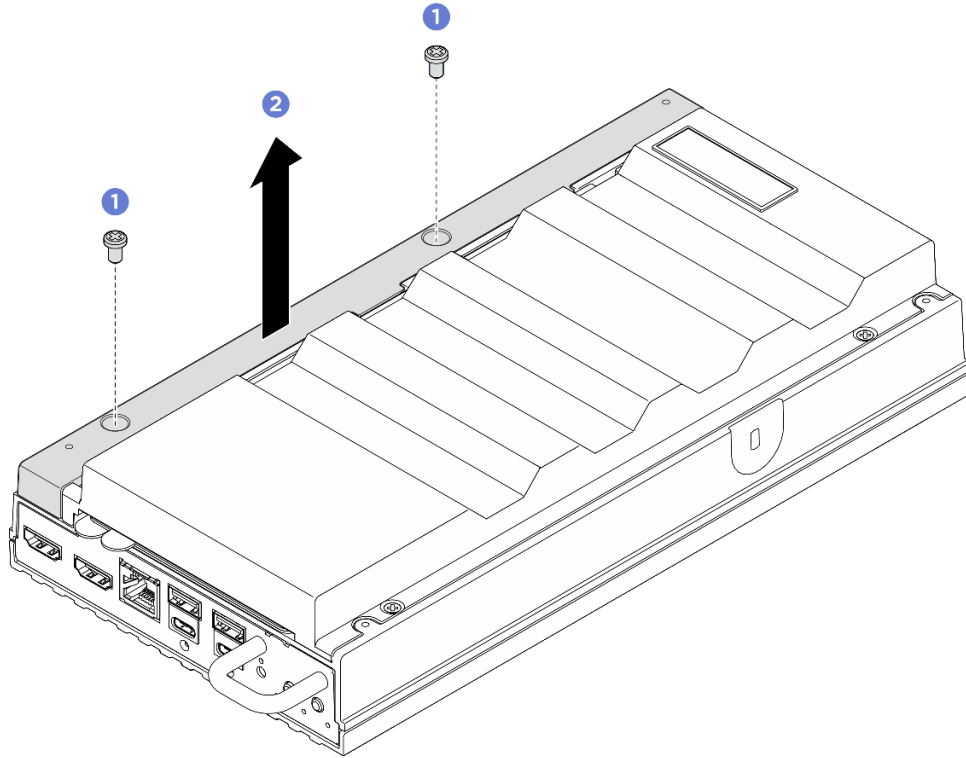
그림 78. 확장 필터 제거
