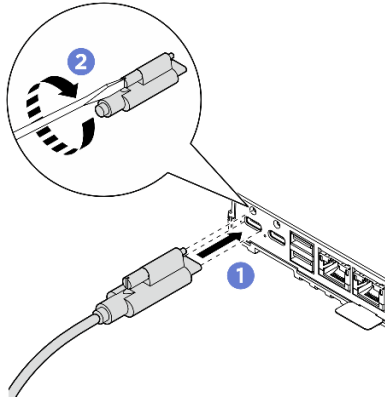
그림 67. 전원 케이블 연결
