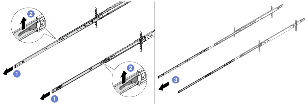
그림 9. 내부 레일 제거
