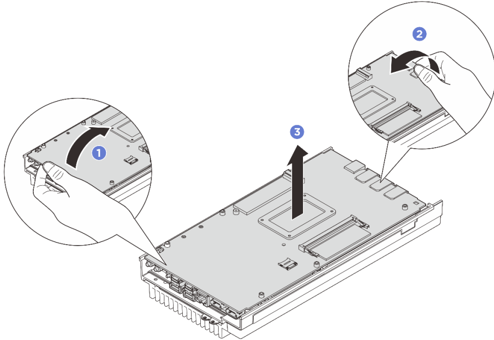
그림 150. 시스템 보드 분해
