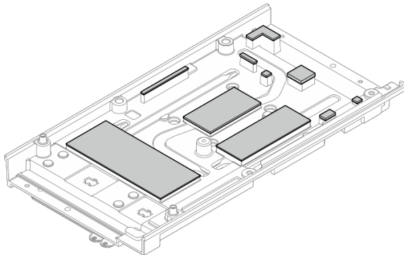
그림 127. 윗면 덮개 열 패드
