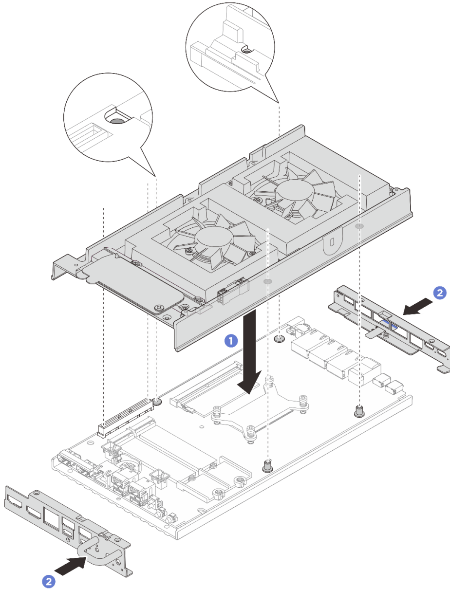
그림 128. 뒷면 덮개 설치
