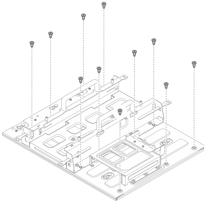
그림 29. 확장 키트를 사용하지 않고 노드 슬리브 제거
