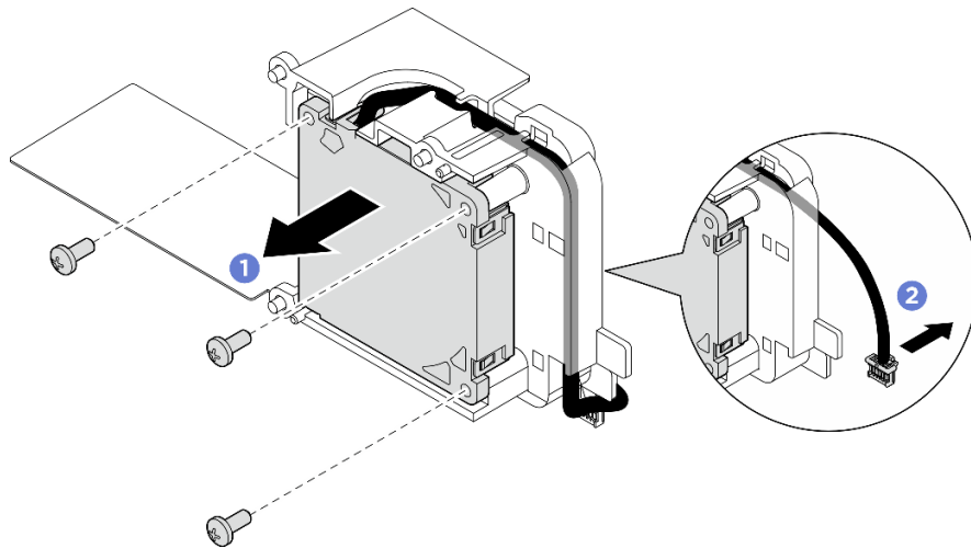
그림 168. 팬 5 제거
