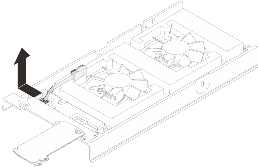
그림 83. 팬 브리지 케이블 제거
