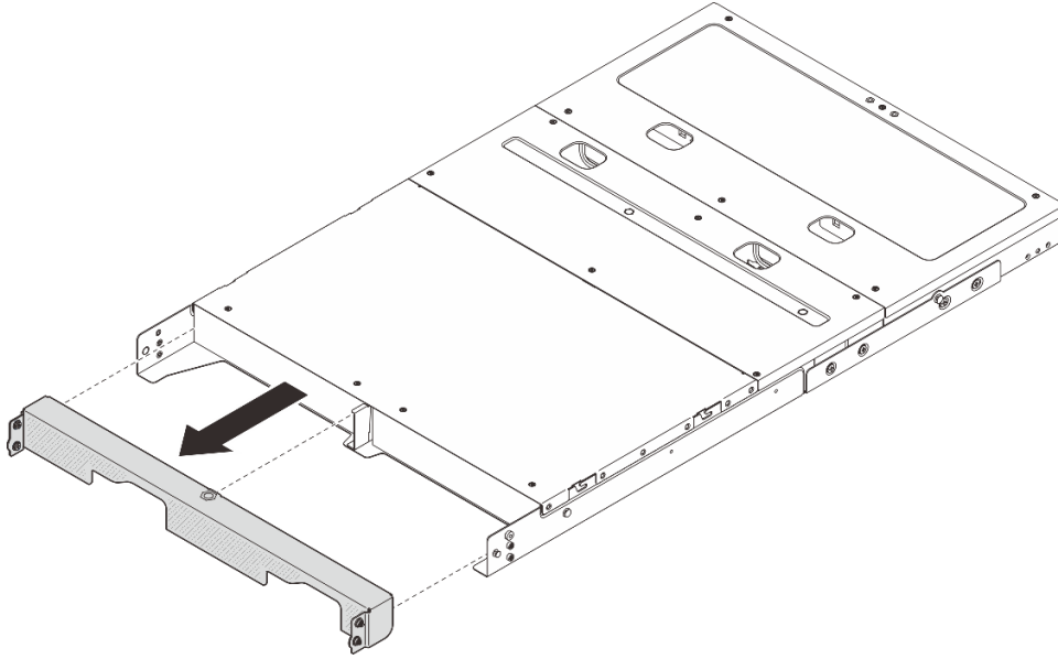
그림 6. 운반 브래킷 제거
