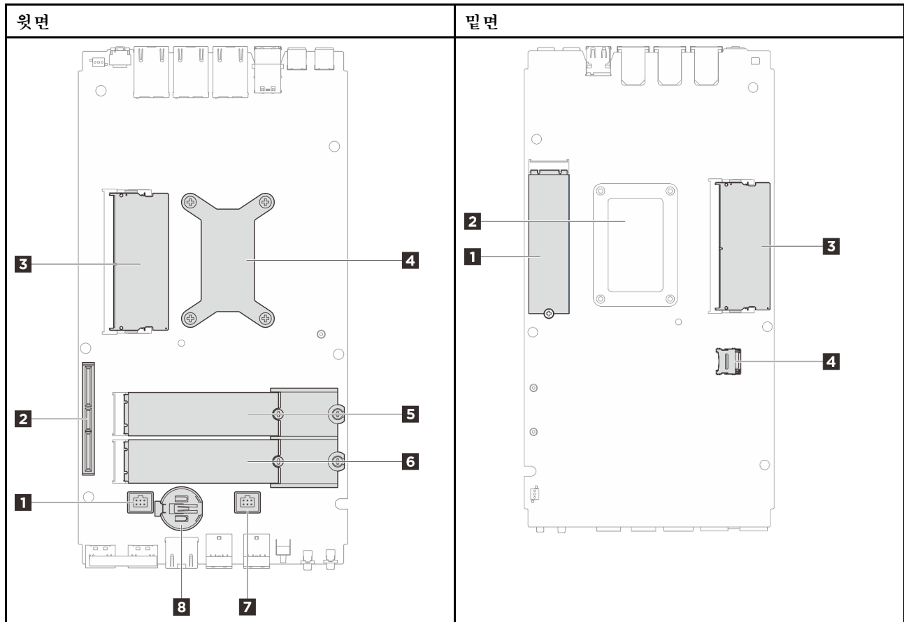
그림 181. 시스템 보드 커넥터
