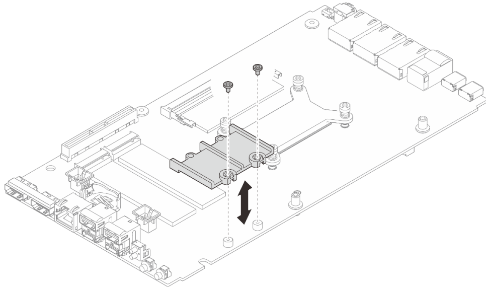
그림 112. M.2 홀더 제거
