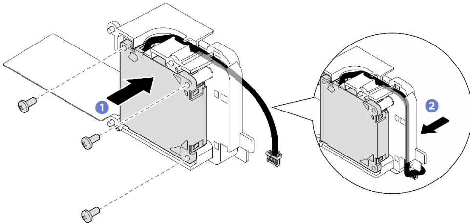
그림 170. 팬 5 설치
