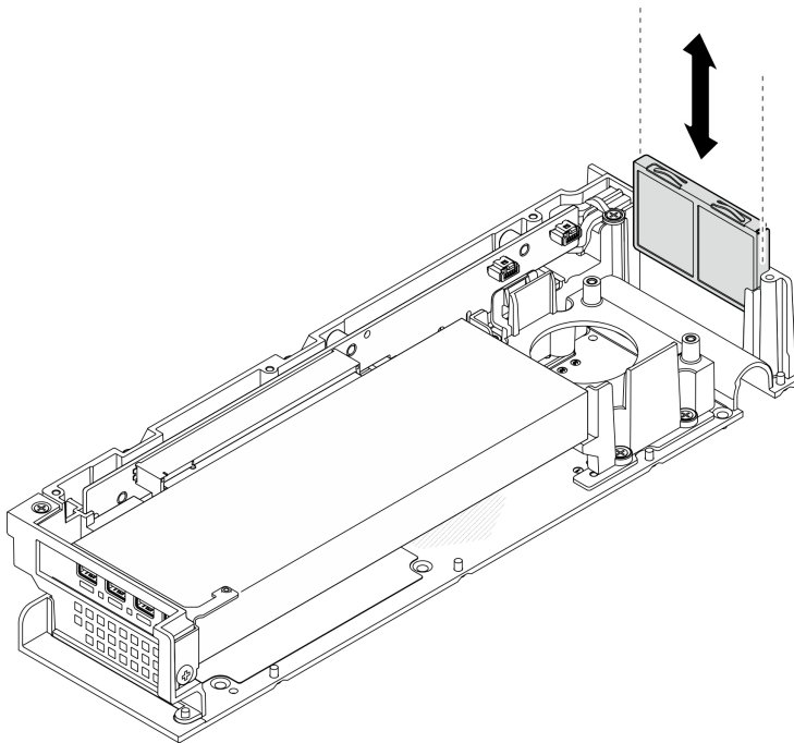
그림 161. 먼지 필터 홀더 설치
