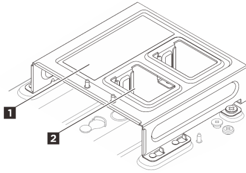
그림 65. 전원 어댑터 슬롯 번호 지정
