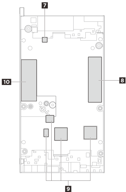
그림 3. 밑면 덮개 - 열 패드 키트 식별 및 위치
