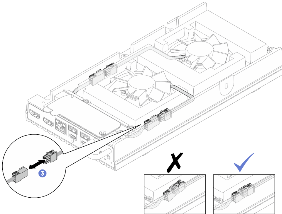
그림 103. 팬 브리지 케이블 연결
