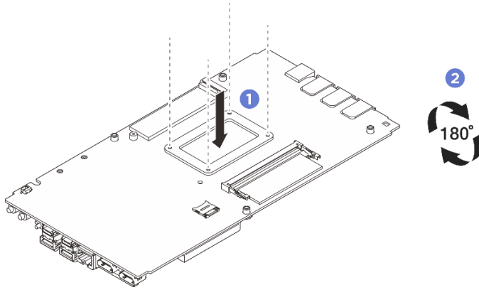
그림 142. 프로세서 백플레이트 설치
