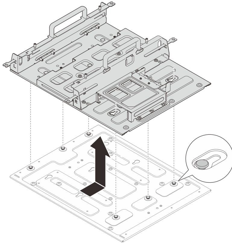
그림 24. 노드 슬리브 제거
