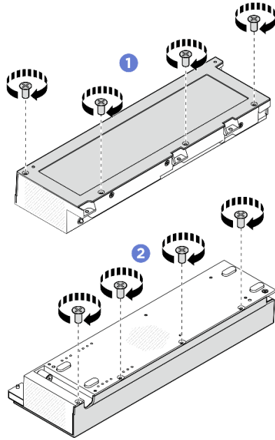
그림 165. 확장 뒷면 덮개 설치
