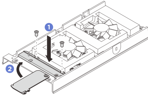
그림 87. 팬 브리지 케이블 덮개 설치
