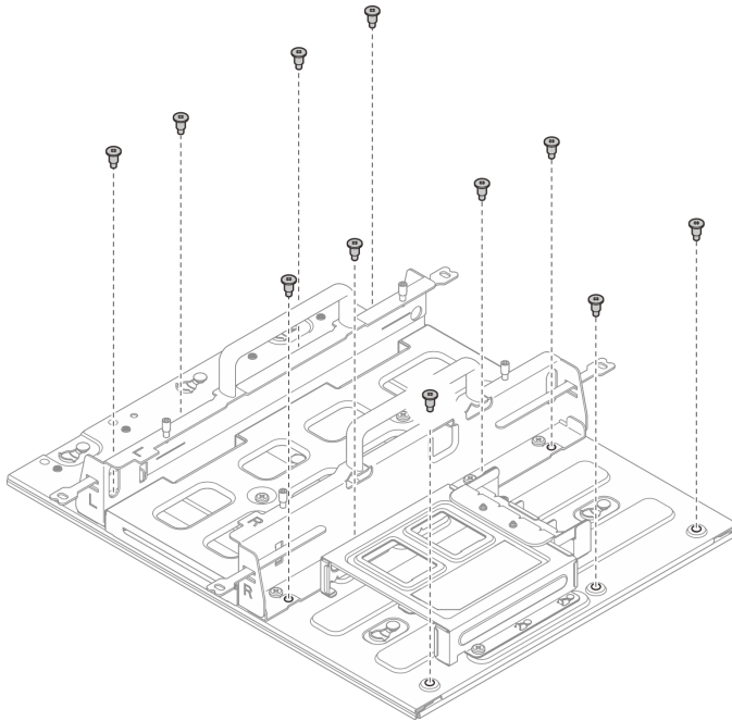
그림 23. 확장 키트를 사용하지 않고 노드 슬리브 제거
