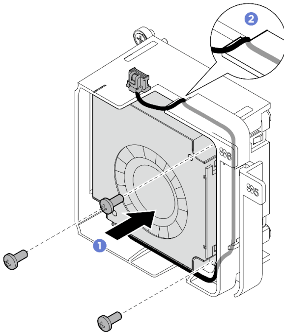
그림 171. 팬 6 설치
