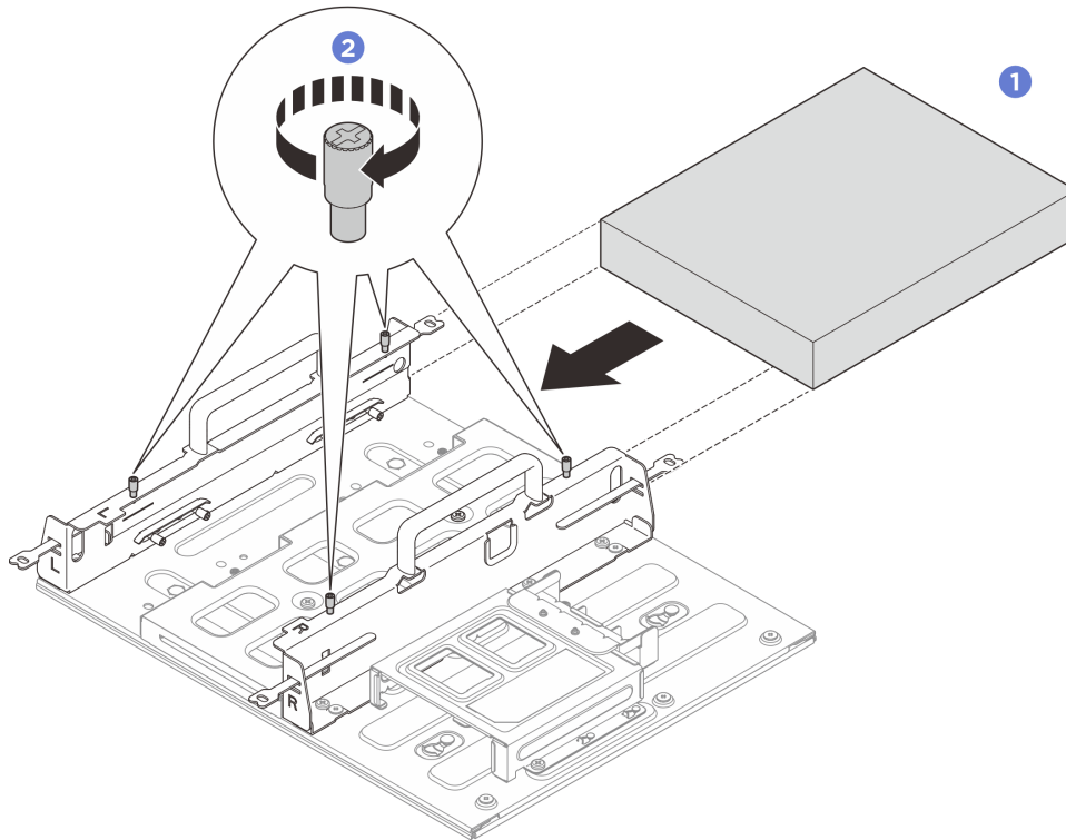
그림 38. 노드 슬리브에 노드 설치
