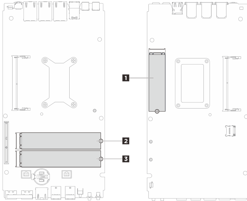
그림 104. M.2 드라이브 슬롯 번호 지정
