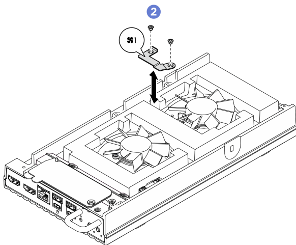
그림 97. 팬 1 브래킷의 나사 위치
