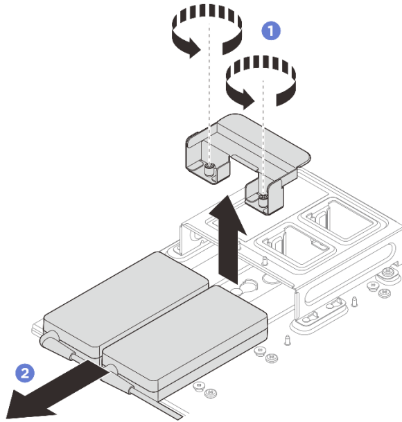
그림 62. 전원 어댑터 제거
