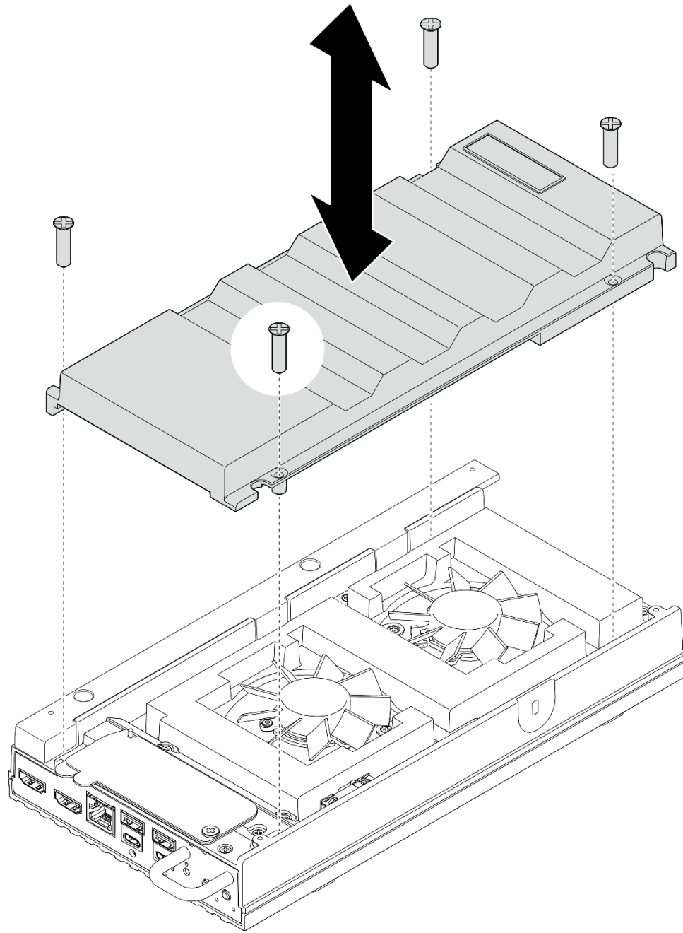
그림 93. 팬 슈라우드 설치
