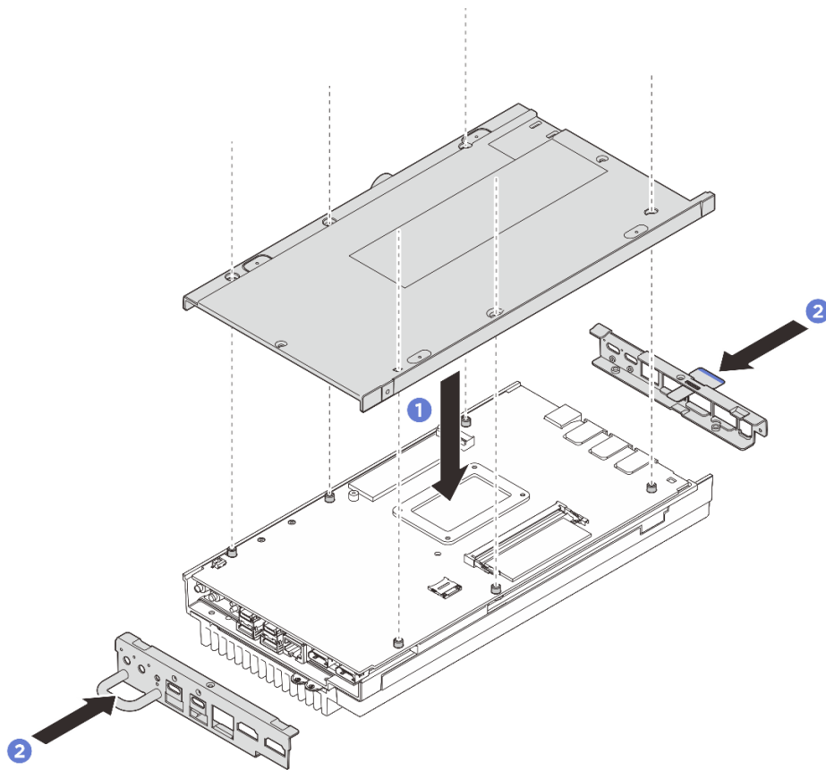
그림 155. 밀면 덮개 설치
