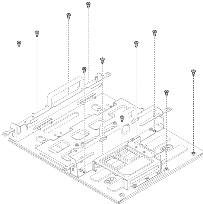
그림 45. 확장 키트를 사용해 노드 슬리브 제거
