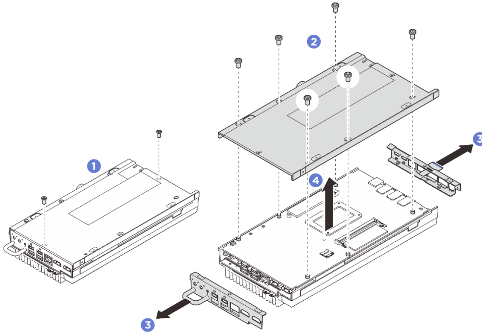
그림 149. 밑면 덮개 제거
