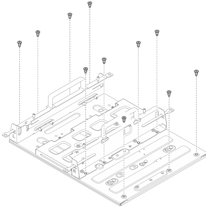
그림 51. 확장 키트를 사용해 노드 슬리브 설치
