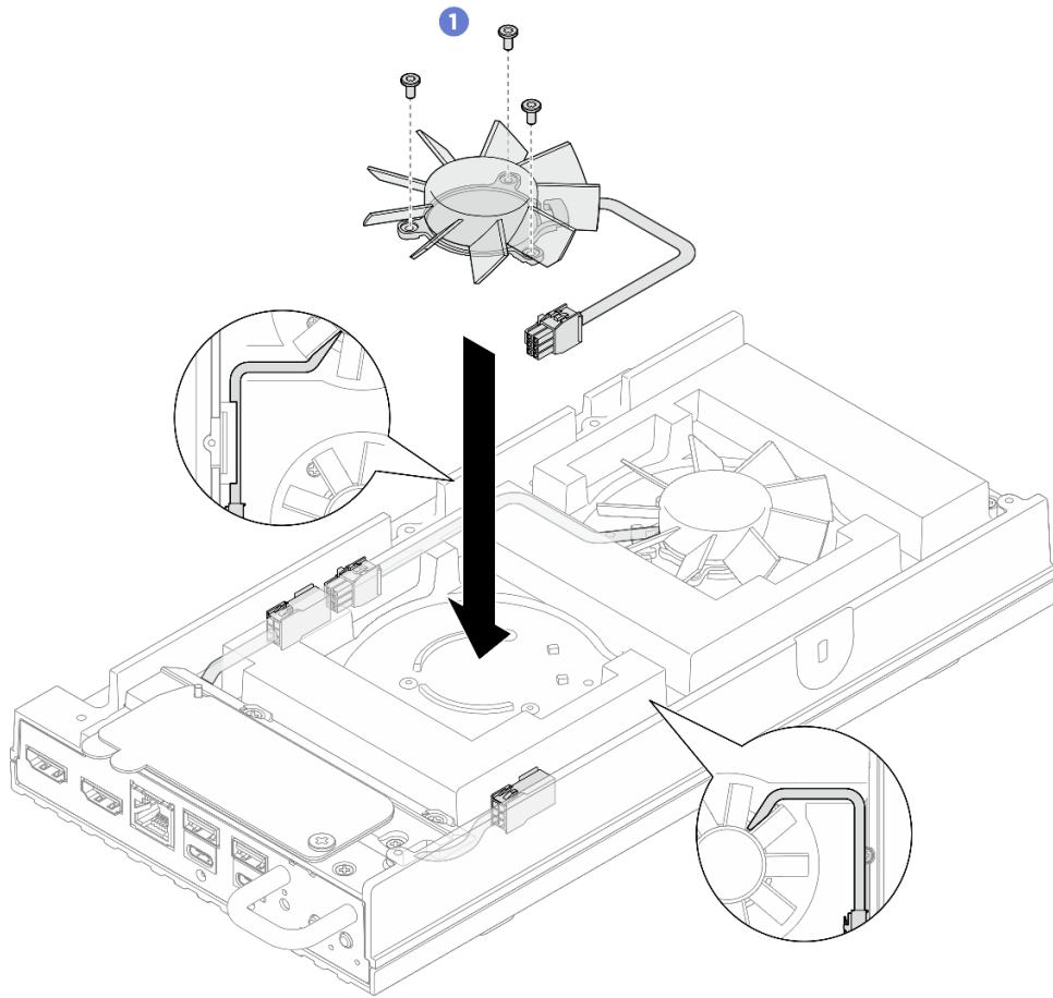
그림 100. 팬 모듈 설치
