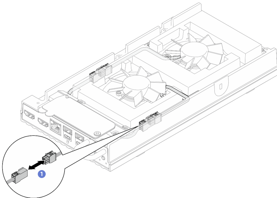
그림 96. 팬 브리지 케이블 분리
