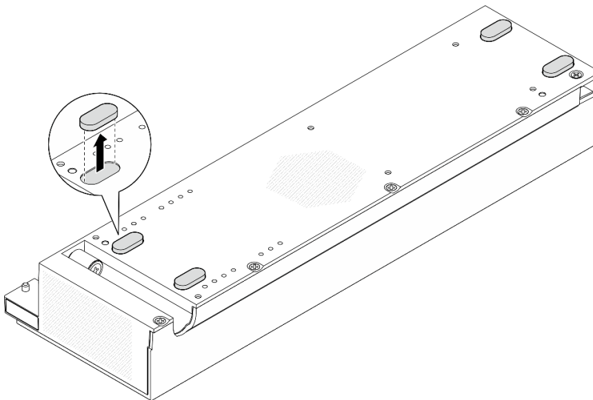
그림 55. PCIe 확장 키트에서 고무 발 제거
