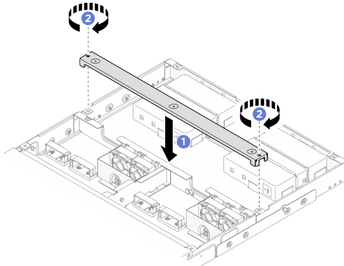
그림 73. 크로스바 설치
