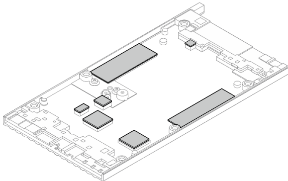
그림 133. 밀면 덮개 열 패드
