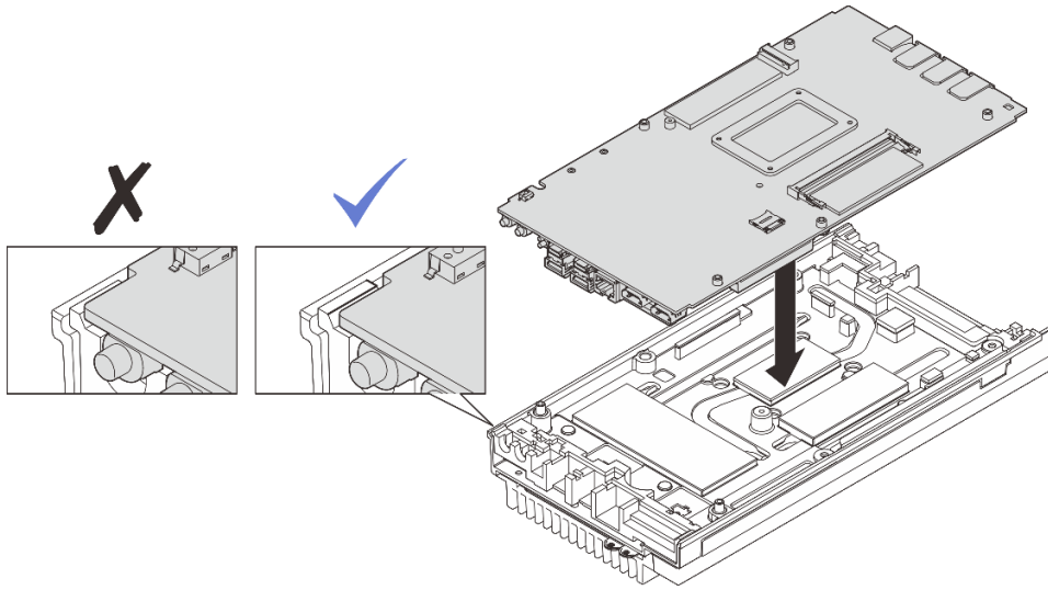
그림 144. 시스템 보드 설치
