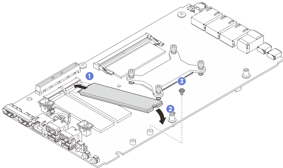
그림 113. M.2 드라이브 유형 22110 설치
