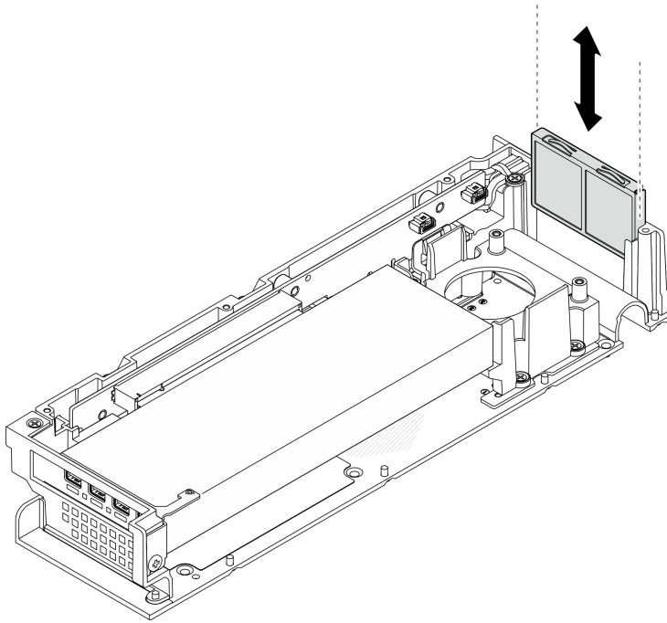
그림 158. 먼지 필터 홀더 제거
