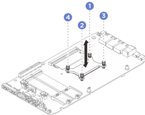
그림 139. 프로세서 방열판 제거
