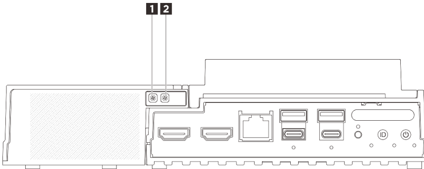
그림 182. 이더넷 어댑터 확장 키트 LED
