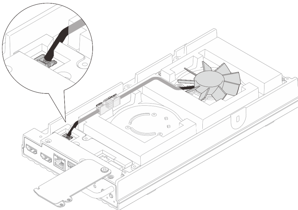
그림 85. 팬 커넥터 1의 케이블 배선
