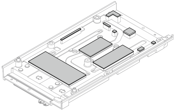
그림 151. 윗면 덮개 열 패드
