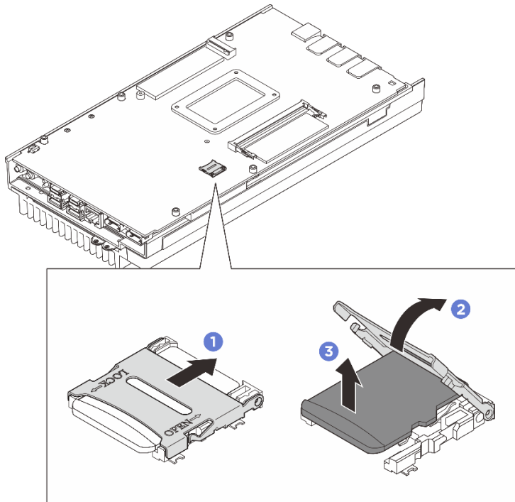
그림 122. MicroSD 카드 제거
