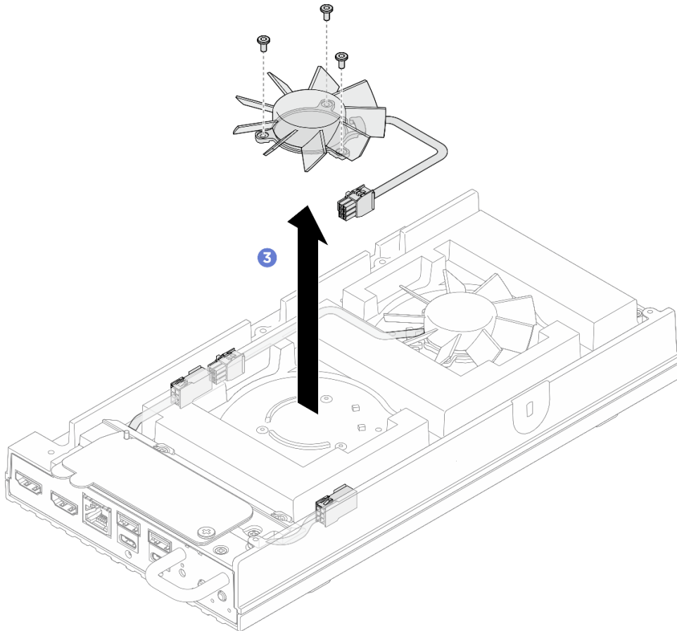
그림 99. 팬 모듈 제거
