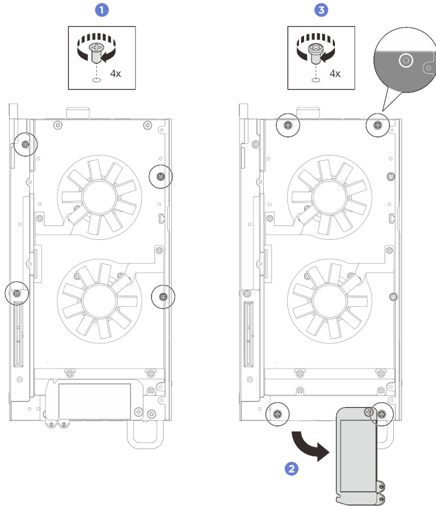
그림 157. 나사 설치
