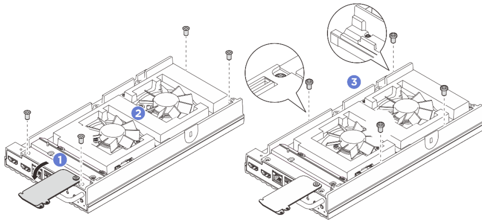
그림 148. 윗면 덮개에서 나사 제거
