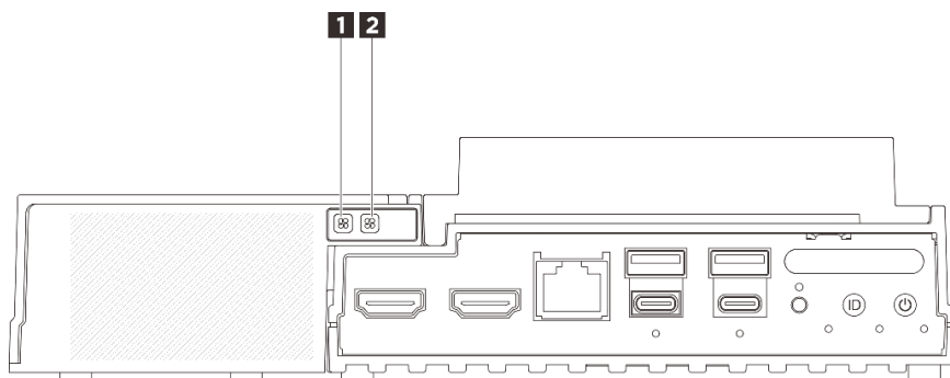
그림 12. 이더넷 어댑터 확장 키트 LED
