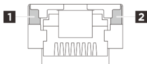
그림 20. 1GbE RJ-45 LAN 포트 링크 및 활동 LED
