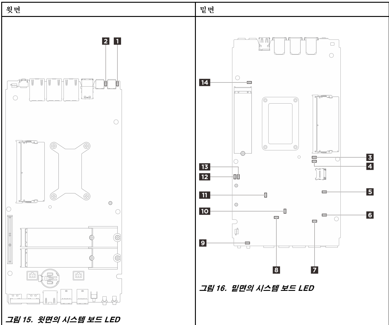
그림 17. 시스템 보드 LED
