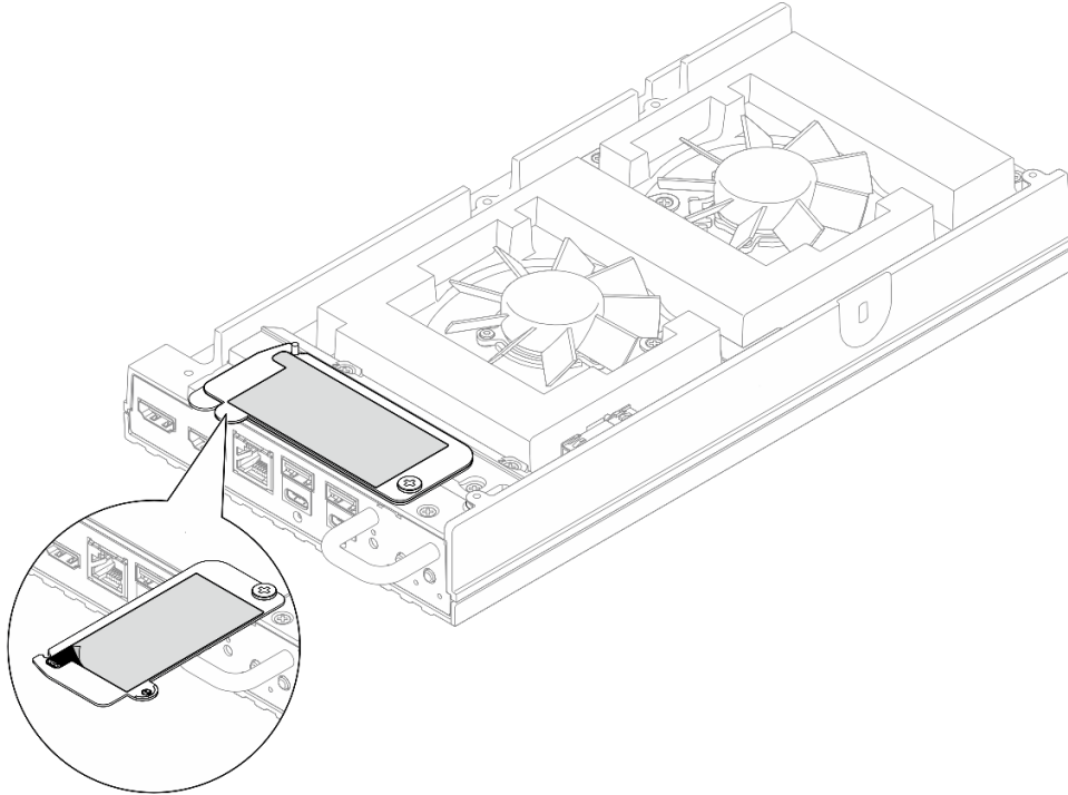
그림 23. 탈착식 정보 탭에 있는 Lenovo XClarity Controller 네트워크 액세스 레이블
