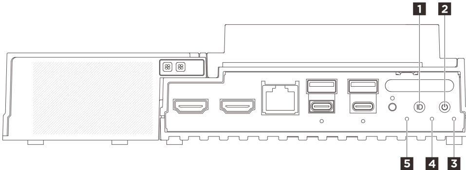
그림 13. 앞면 LED
