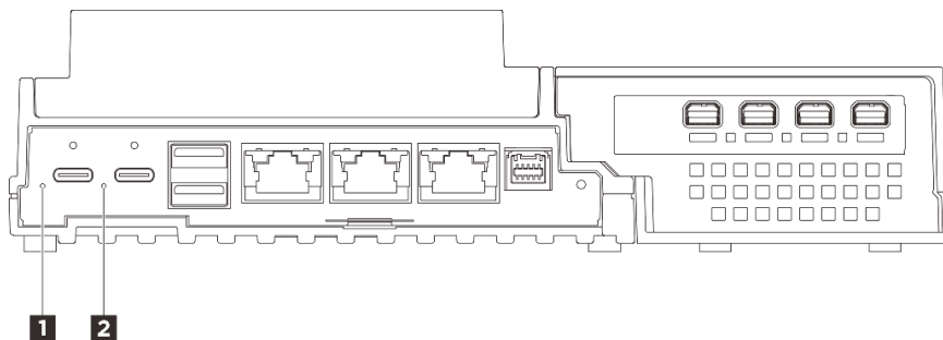
그림 14. 뒷면 LED
