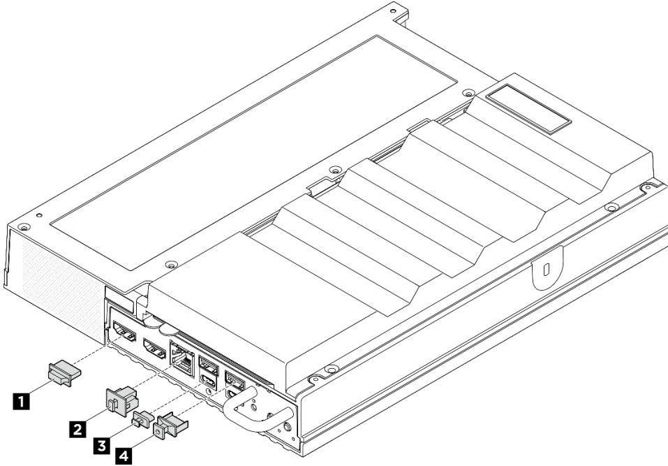
그림 4. 앞면 I/O 필터
