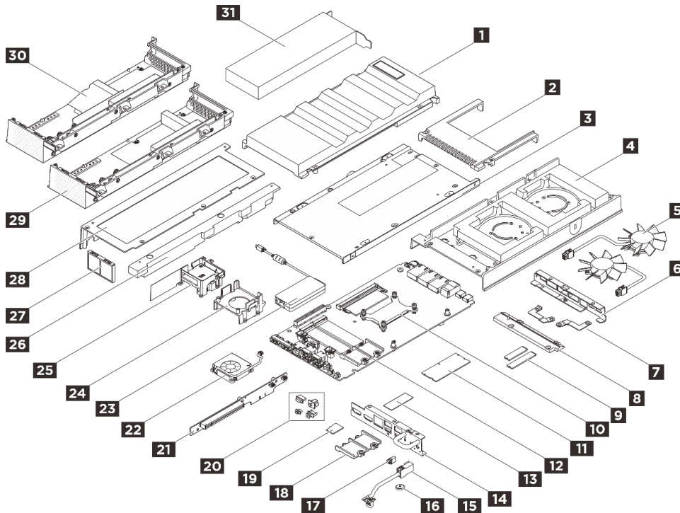
그림 21. 서버 구성 요소
