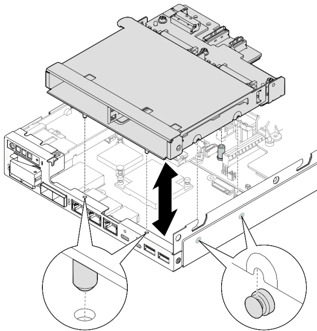
Figure 62. Retrait du boîtier d'unités de disque dur
