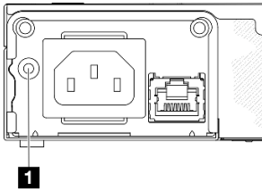
Figure 154. Voyant d'état PMB, entrée d'alimentation en courant alternatif
