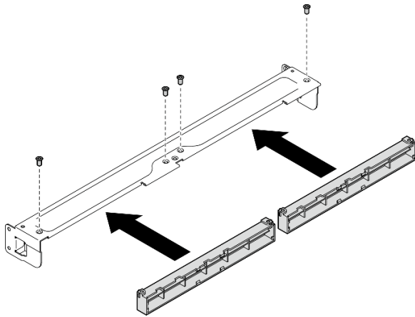
Figure 19. Installation d'un support de filtre anti-poussière
