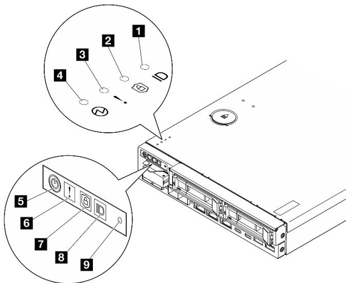
Figure 146. Voyants du panneau opérateur avant
