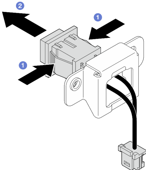
Figure 81. Retrait du commutateur de verrou avec câble du support
