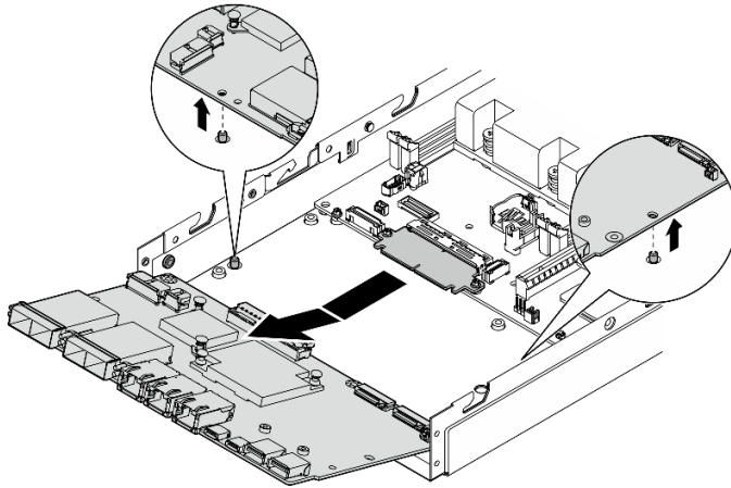
Figure 113. Retrait de la carte de module d'E/S
