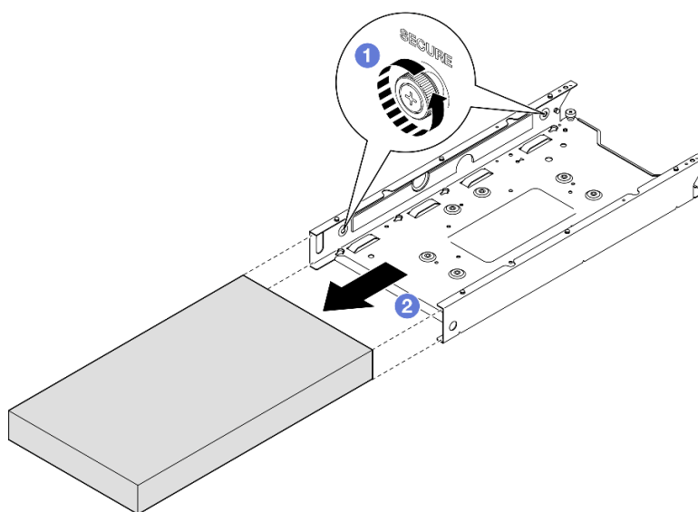
Figure 32. Retrait d'un nœud d'un manchon de nœud
