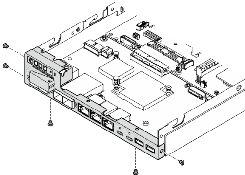
Figure 128. Installation des vis du panneau d'E/S avant
