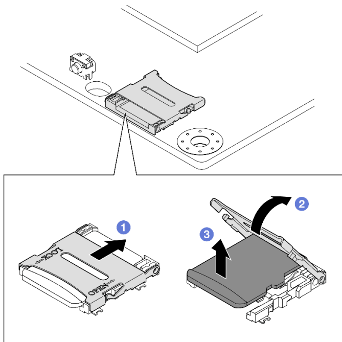
Figure 94. Retrait d'une carte MicroSD
