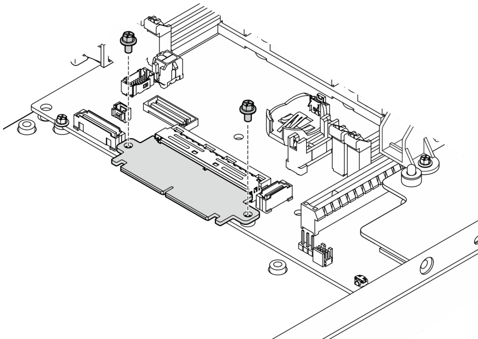
Figure 124. Installation des vis de la carte passerelle
