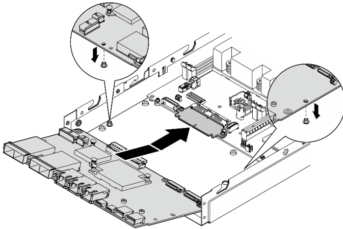
Figure 125. Installation de la carte de module d'E/S
