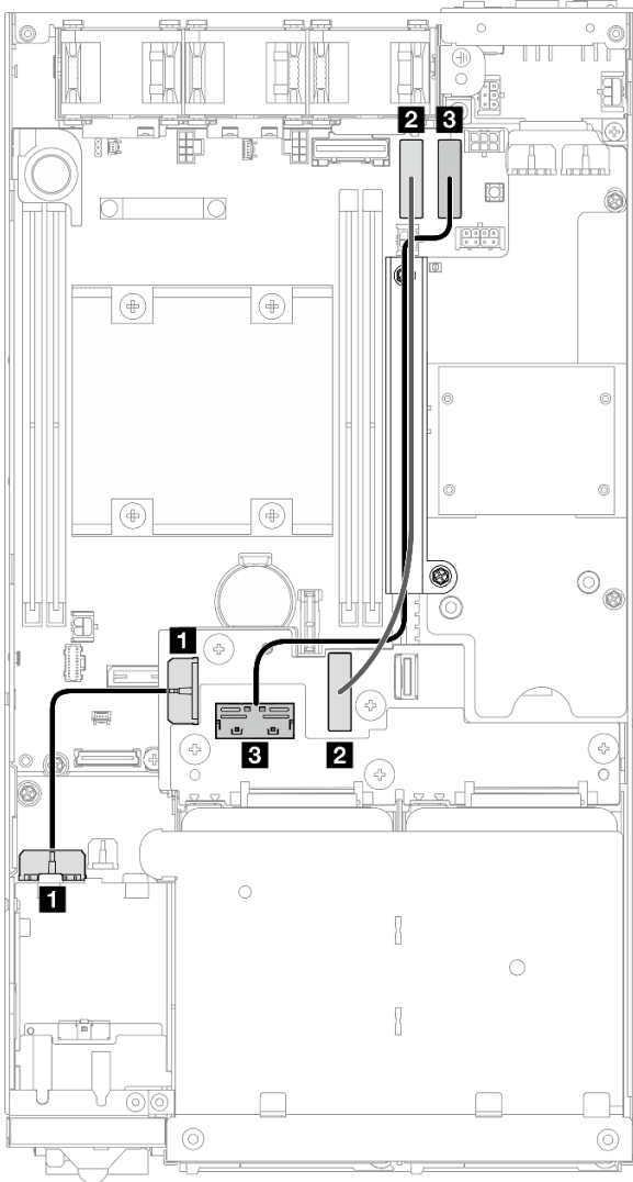
Figure 137. Câble d'alimentation du fond de panier et câbles haut débit Gen 4 pour les unités de 7 mm ; Fond de panier d'unité 1 (inférieur) et Fond de panier d'unité 2 (supérieur)
