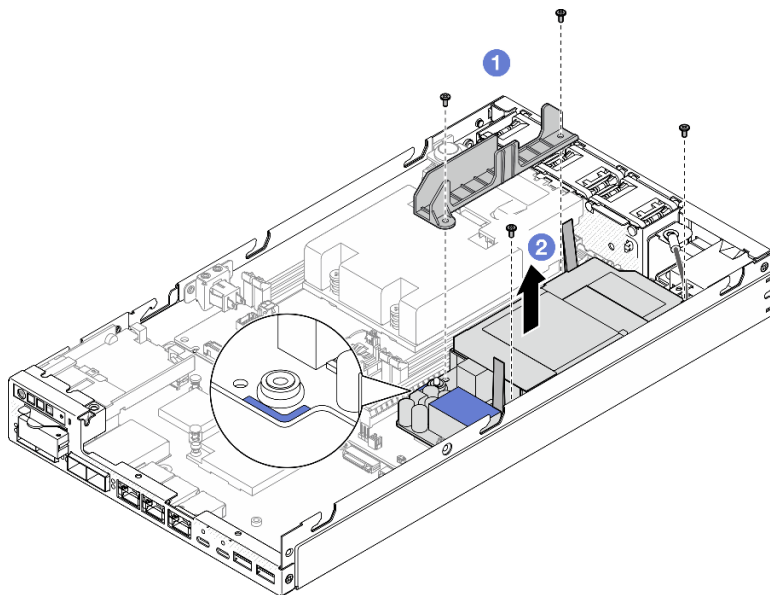
Figure 74. Retrait du support de câbles et de l'alimentation interne
