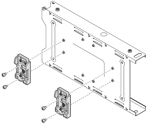
Figure 25. Retrait des clips de rail DIN du manchon de nœud
