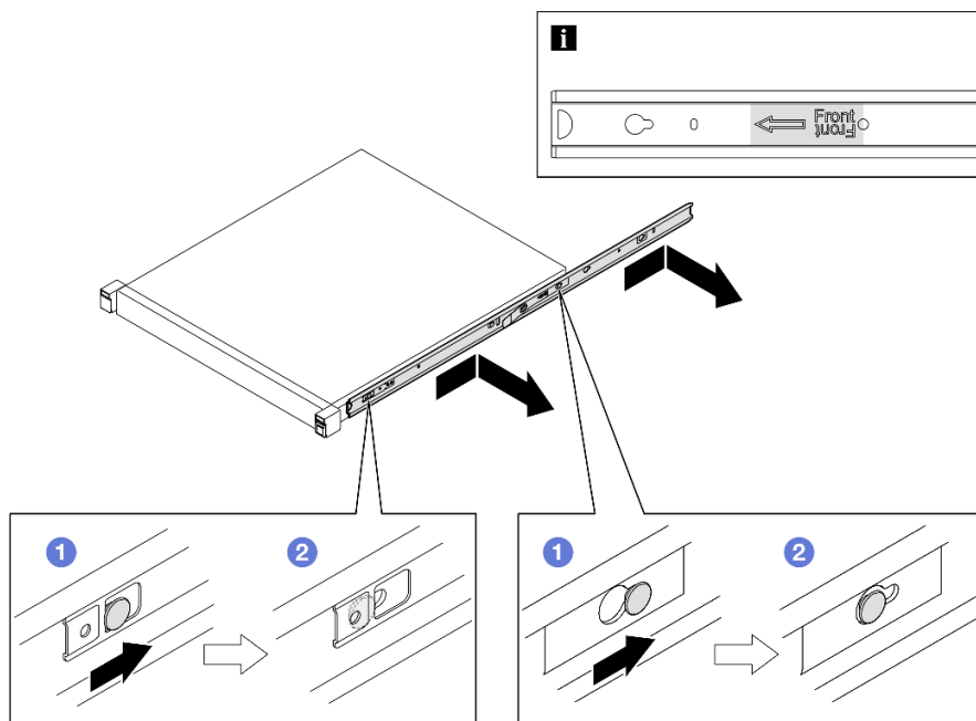
Figure 7. Retrait des glissières internes
