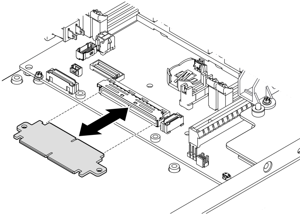
Figure 123. Installation de la carte passerelle
