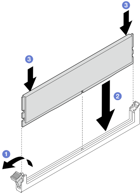
Figure 93. Installation d'un module de mémoire
