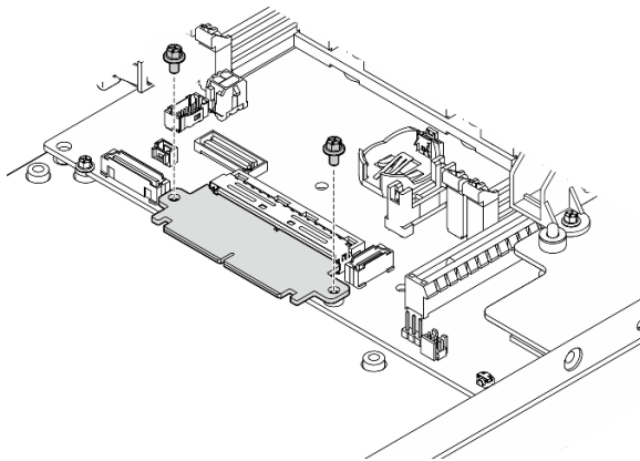
Figure 114. Retrait des vis de la carte passerelle
