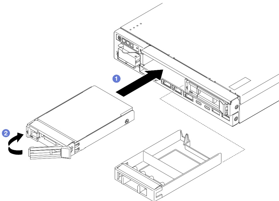
Figure 69. Installation d'une unité remplaçable à chaud
