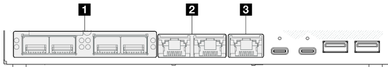
Figure 147. Voyants de port LAN du Module d'E/S 10/25 GbE
