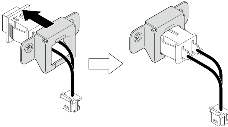
Figure 82. Installation du commutateur de verrou avec câble sur le support
