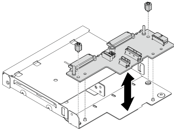
Figure 64. Retrait du Fond de panier d'unité 1 (inférieur)
