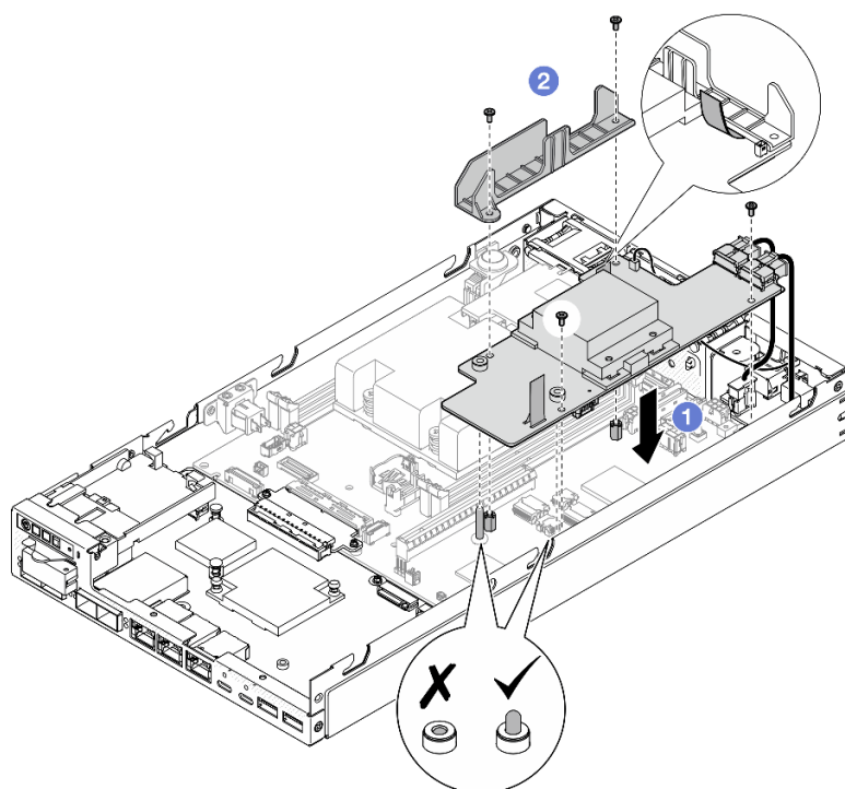
Figure 104. Installation de la carte de module d'alimentation
