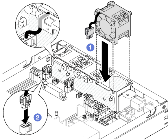
Figure 71. Installation d'un module ventilateur
