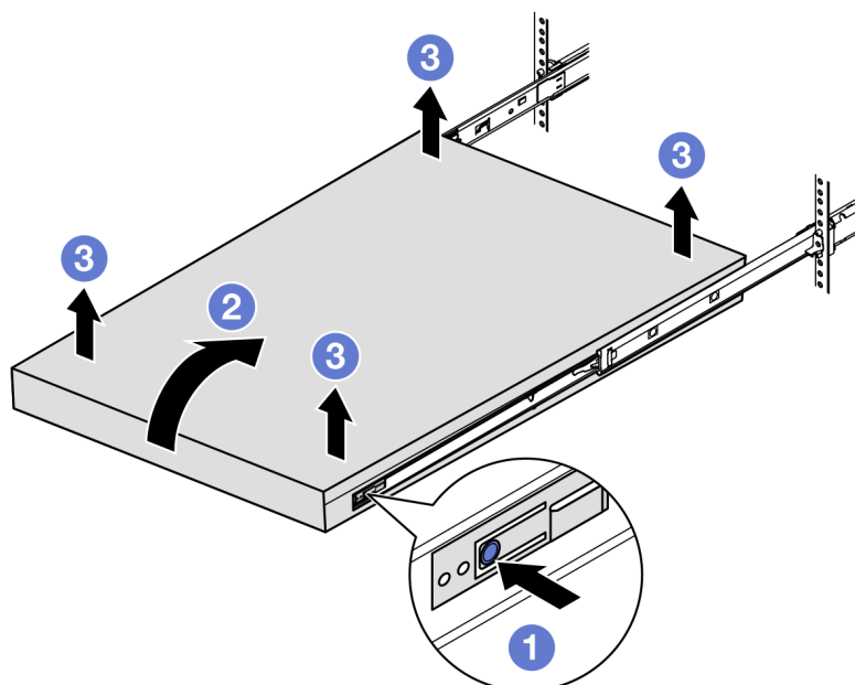
Figure 8. Retrait du boîtier de l'armoire en le soulevant
