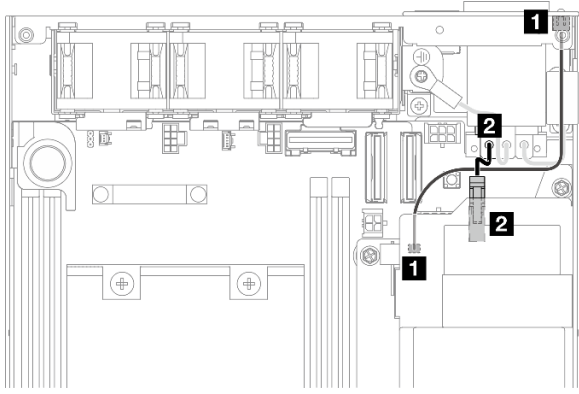
Figure 141. Acheminement des câbles pour AC PIB et AC PMB
