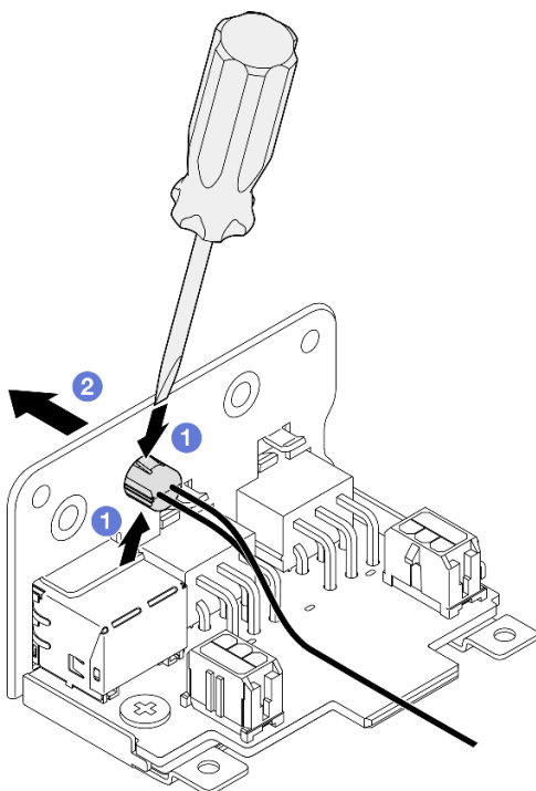
Figure 97. Retrait du câble du voyant d'état PMB du module DC PIB
