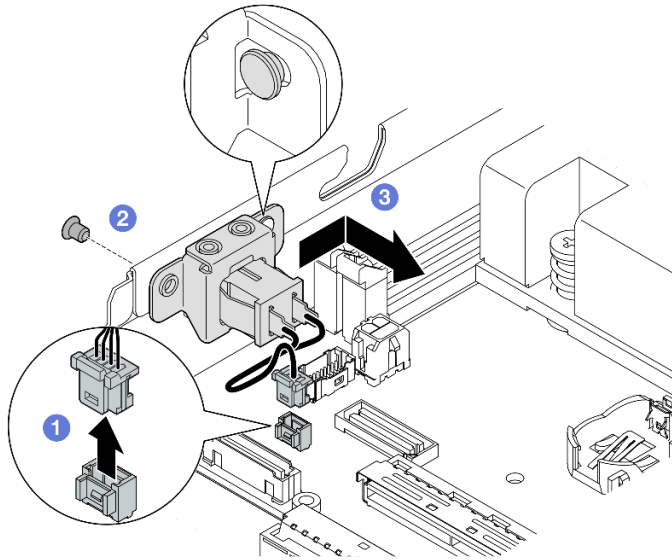
Figure 80. Retrait du commutateur de verrou avec câble
