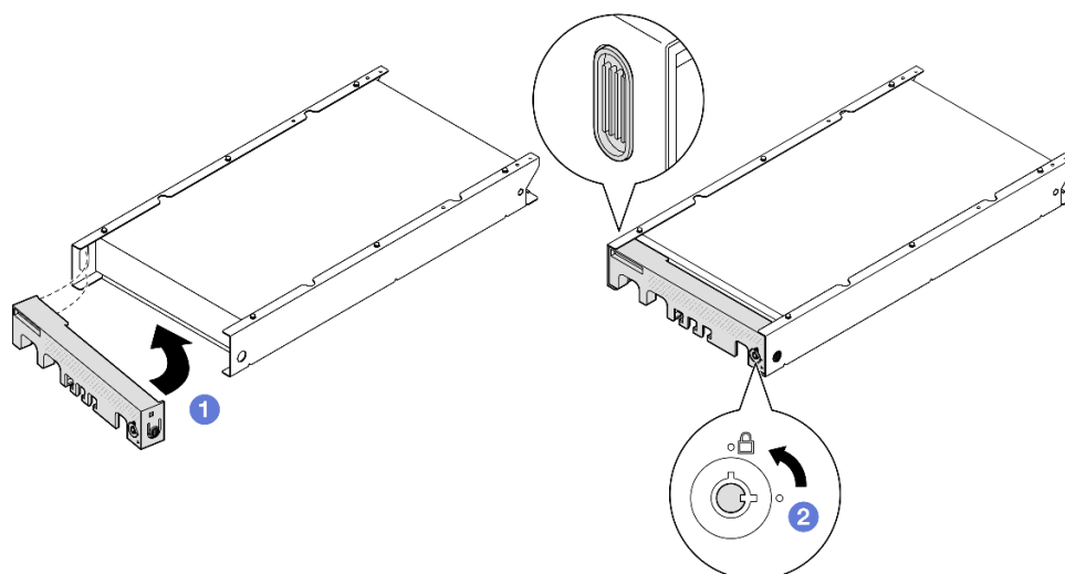
Figure 39. Installation d'un panneau de sécurité sur un manchon de nœud
