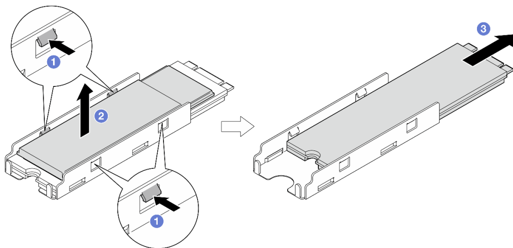
Figure 85. Retrait du dissipateur thermique M.2
