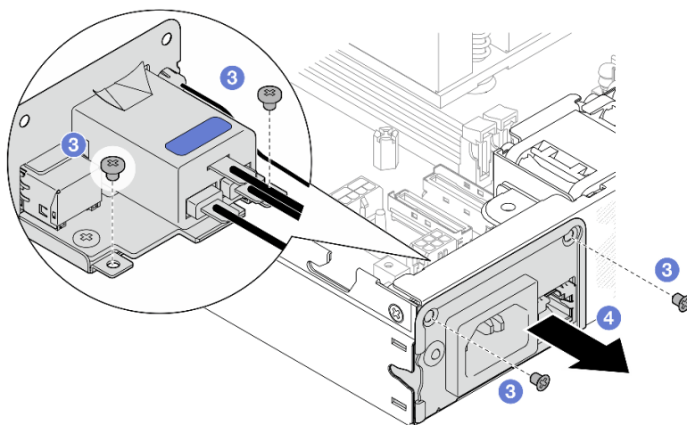
Figure 98. Retrait du module de carte d'entrée d'alimentation
