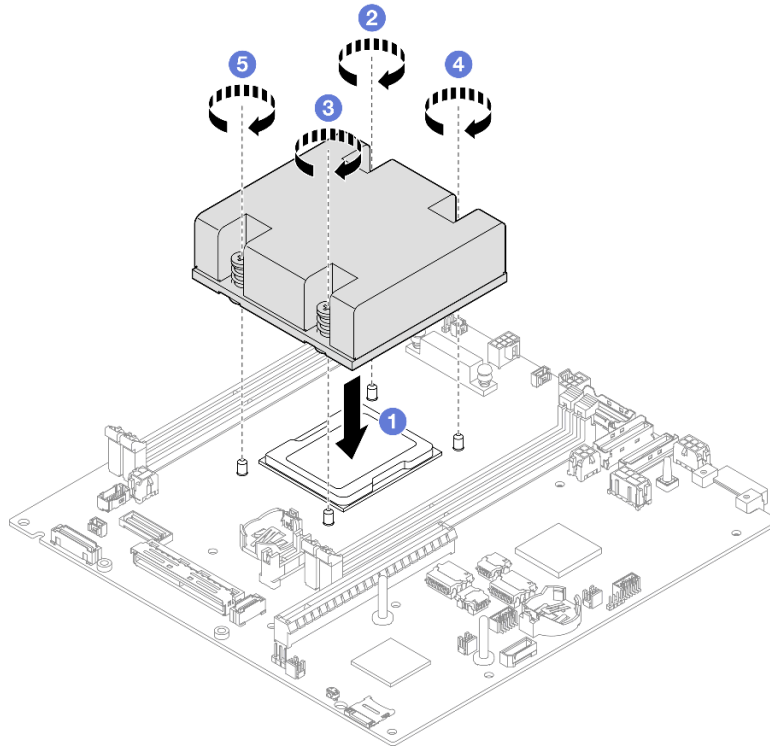
Figure 107. Installation d'un dissipateur thermique de processeur
