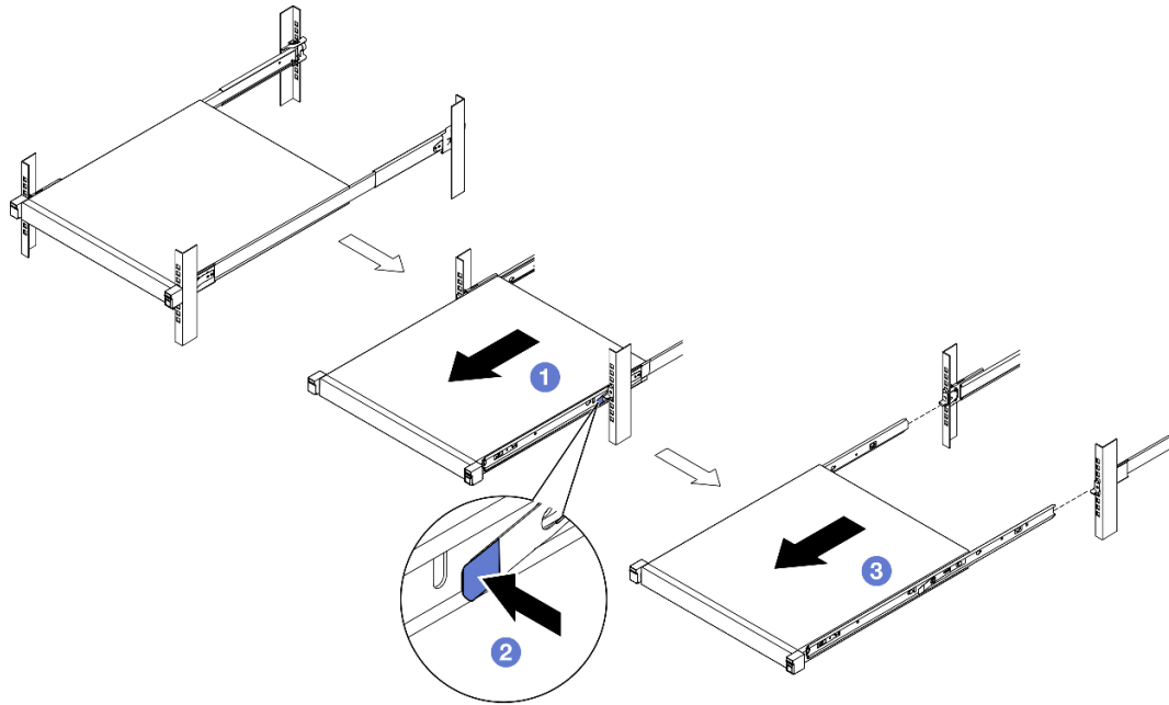
Figure 5. Retrait du boîtier de l'armoire en le faisant glisser
