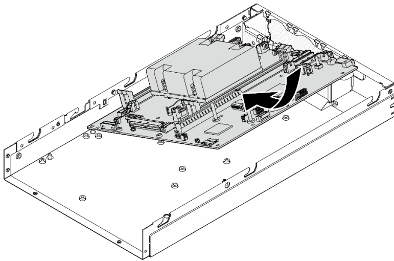
Figure 119. Installation d'une carte mère
