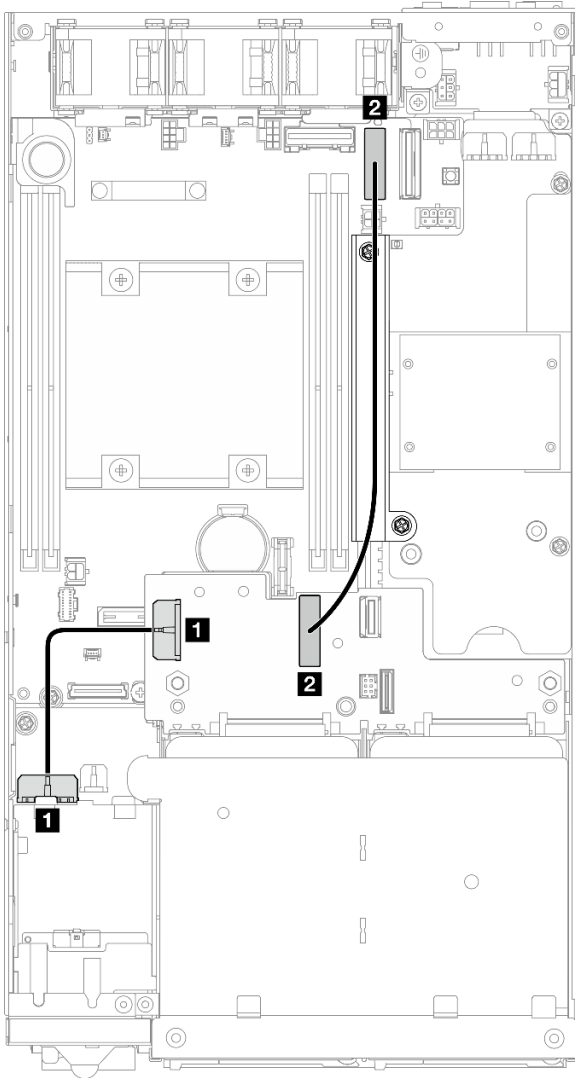
Figure 135. Câble d'alimentation du fond de panier et câble haut débit Gen 4 pour les unités de 15 mm ; Fond de panier d'unité 1 (inférieur)
