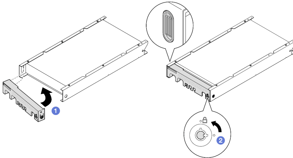
Figure 30. Installation d'un panneau de sécurité sur un manchon de nœud
