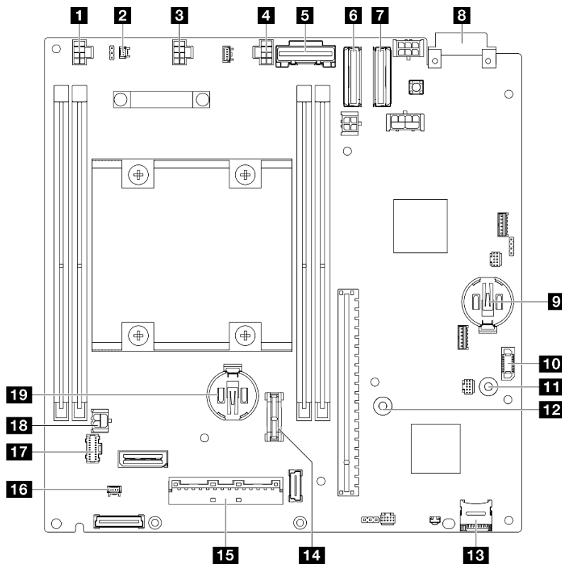
Figure 144. Connecteurs de la carte mère
