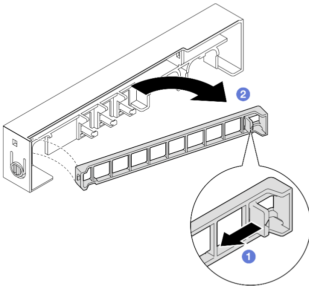
Figure 41. Retrait du support de filtre anti-poussière
