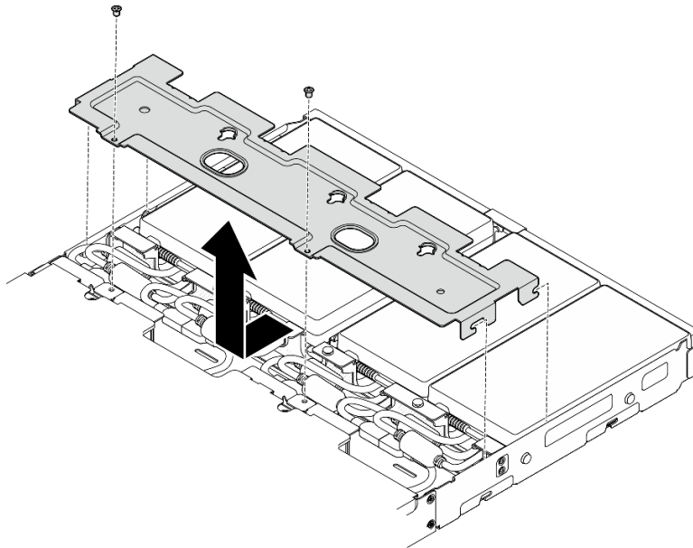
Figure 46. Retrait du couvre-câble d'alimentation, boîtier 1U2N
