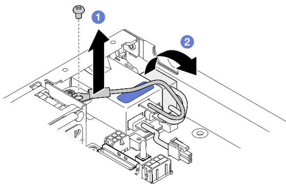
Figure 98. Retrait du module de carte d'entrée d'alimentation
