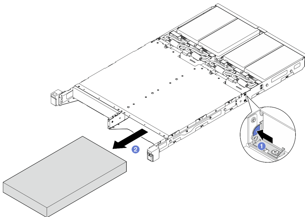
Figure 9. Retrait d'un nœud d'un boîtier 1U2N
