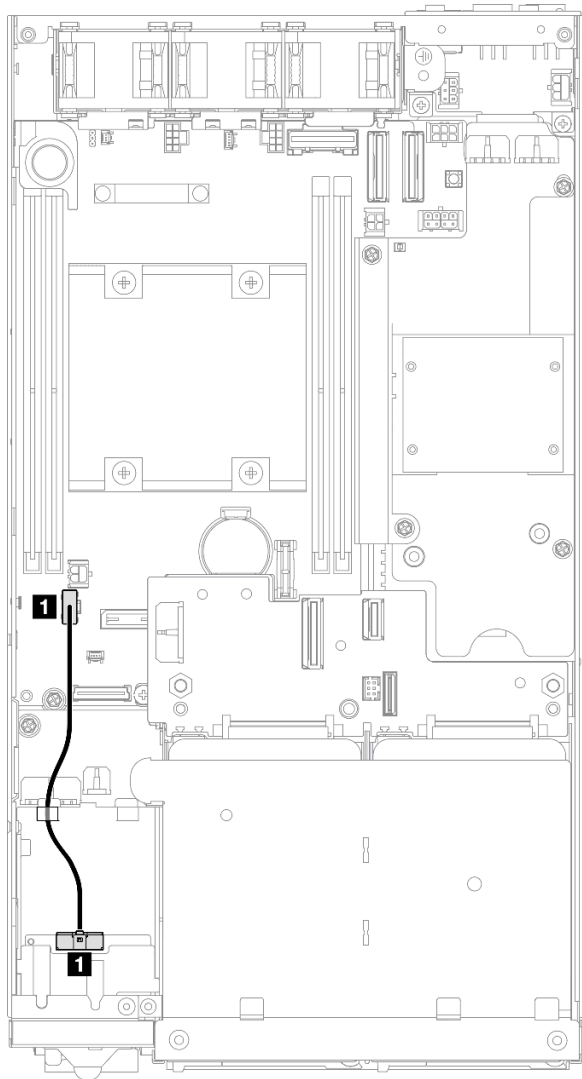
Figure 138. Cheminement des câbles du bloc d'opérateur avant
