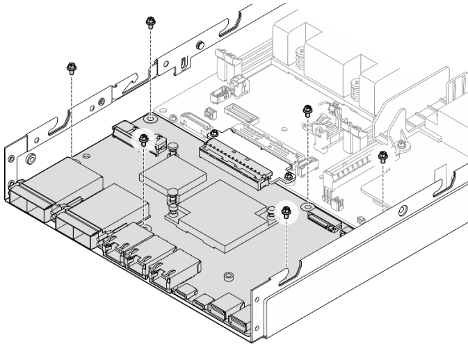
Figure 112. Retrait des vis de la carte de module d'E/S
