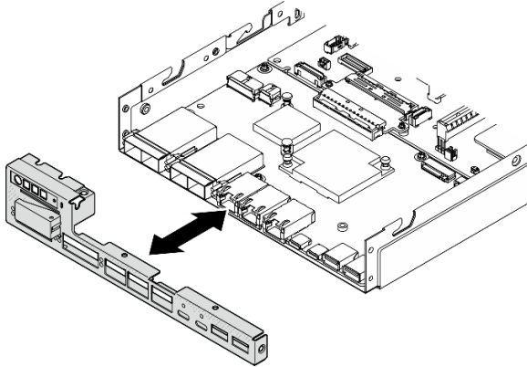
Figure 127. Installation du panneau d'E/S avant
