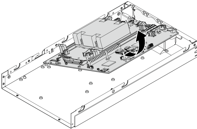
Figure 118. Retrait de la carte mère
