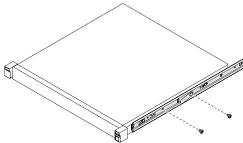
Figure 6. Retrait des vis des glissières internes
