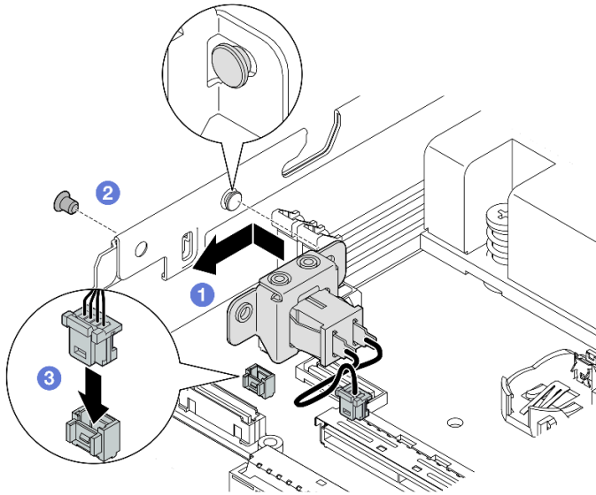
Figure 83. Installation d'un commutateur de verrou avec câble
