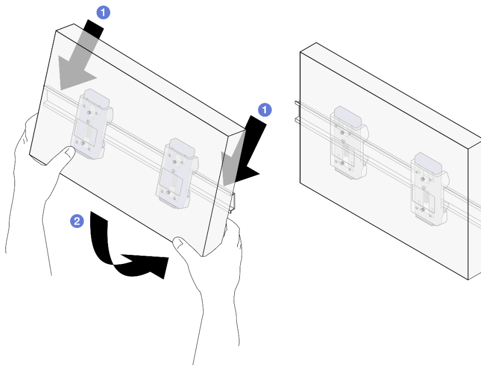
Figure 28. Installation du manchon de nœud sur le rail DIN
