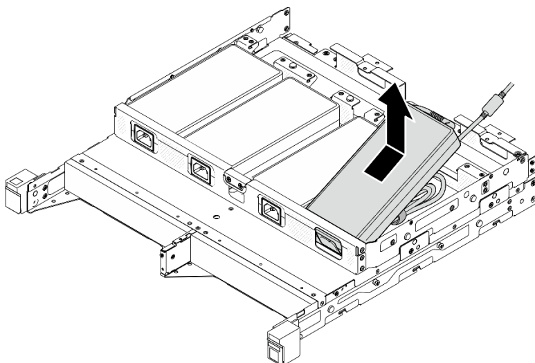
Figure 49. Retrait de l'adaptateur d'alimentation, boîtier 2U2N
