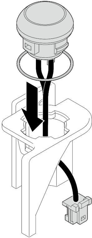
Figure 78. Installation du commutateur d'intrusion avec câble dans le support du commutateur
