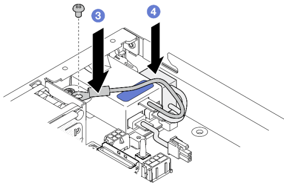
Figure 102. Installation du fil de terre AC PIB et du capuchon en X
