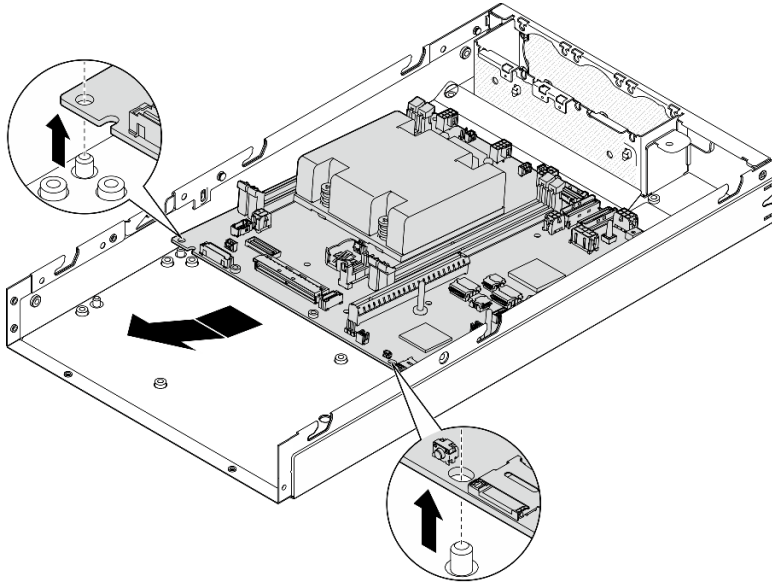
Figure 117. Retrait de la carte mère
