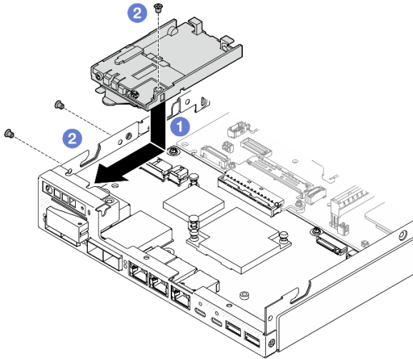
Figure 73. Installation du bloc opérateur avant
