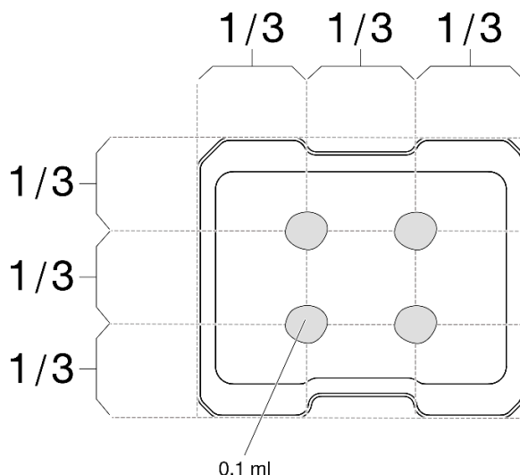
Figure 106. Application de la pâte thermoconductrice
