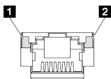
Figure 151. Voyants de Port de gestion système XCC(RJ-45 1 GbE)
