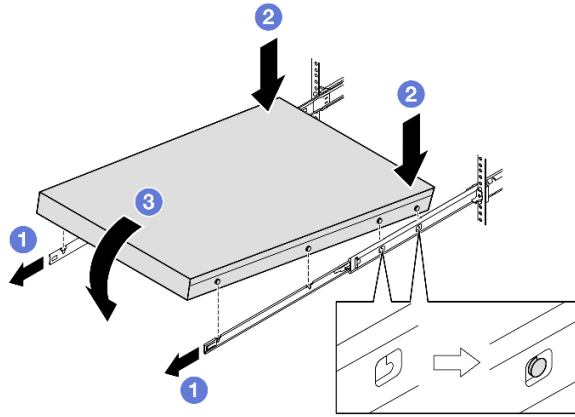
Figure 16. Installation du boîtier dans l'armoire en le tournant
