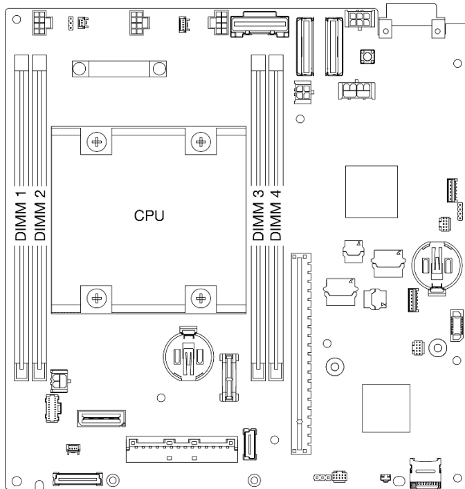
Figure 90. Les emplacements du module de mémoire sur la carte mère
