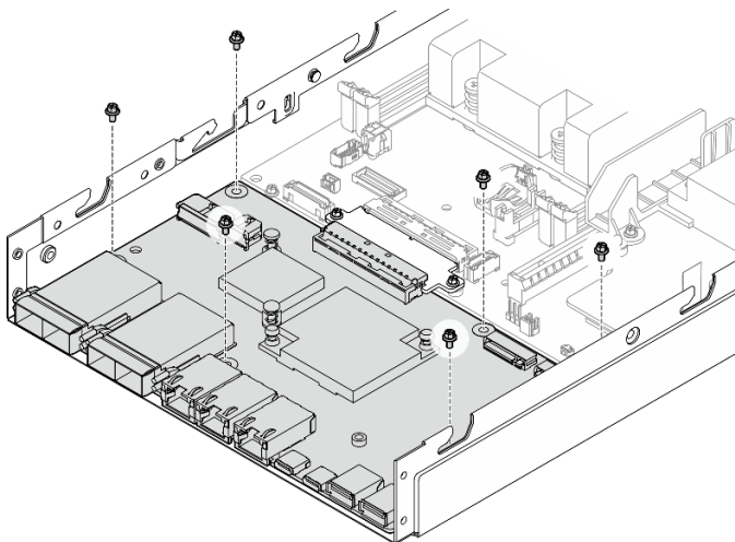
Figure 126. Installation des vis de la carte de module d'E/S
