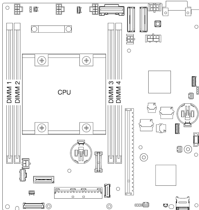
Figure 92. Les emplacements du module de mémoire sur la carte mère
