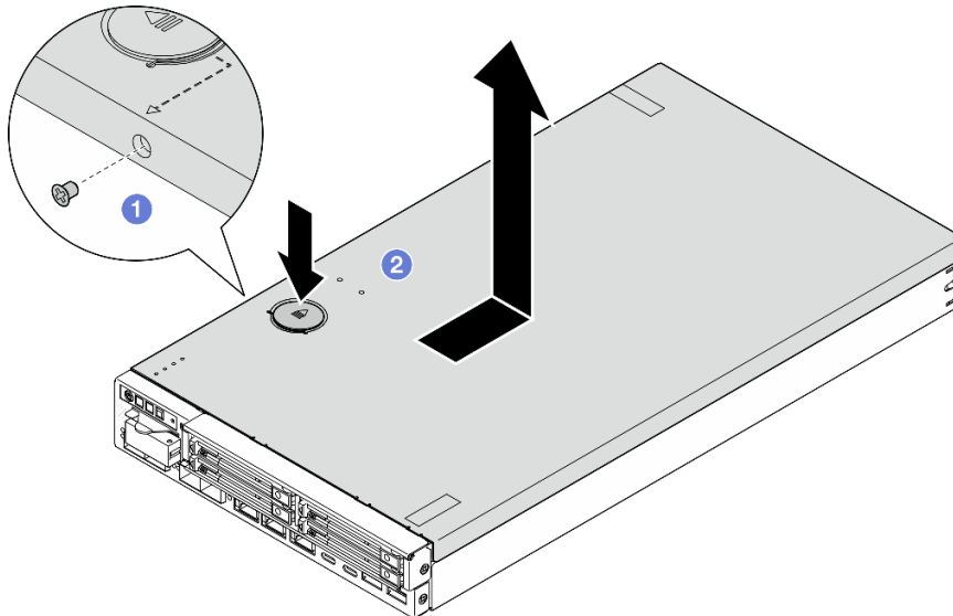
Figure 129. Retrait du carter supérieur
