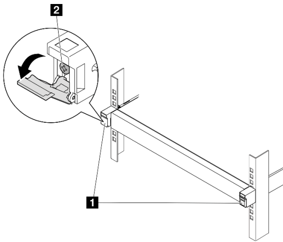
Figure 4. Retrait des vis des loquets de déblocage d'armoire
