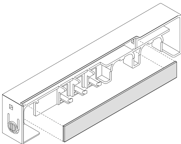
Figure 42. Retrait du filtre anti-poussière du panneau de sécurité
