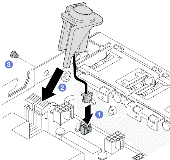
Figure 79. Installation du commutateur de détection d'intrusion avec câble sur le nœud
