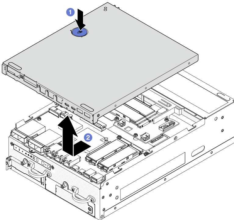
Figura 191. Extracción de la cubierta inferior
