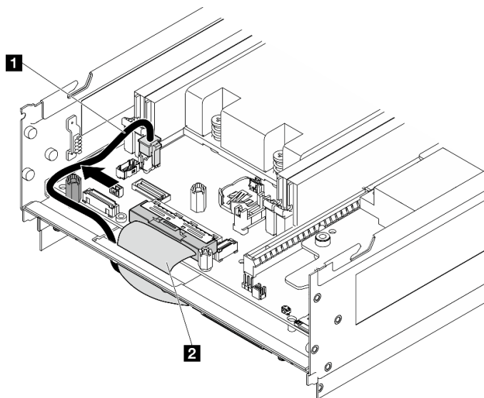
Figura 276. Disposición de los cables de la placa de E/S
