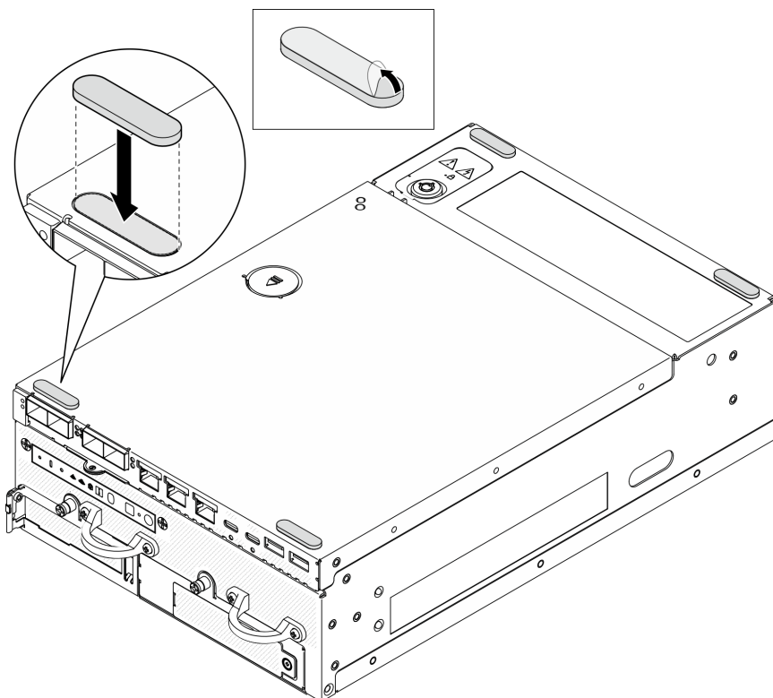
Figura 271. Instalación de las patas de goma
