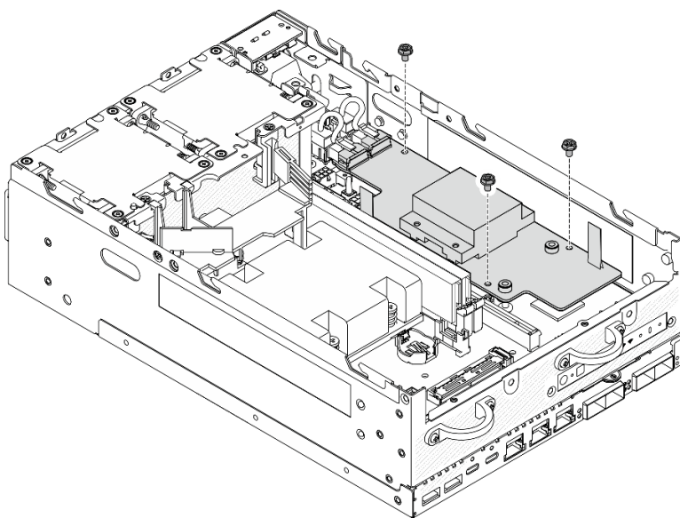
Figura 209. Aflojado de los tornillos
