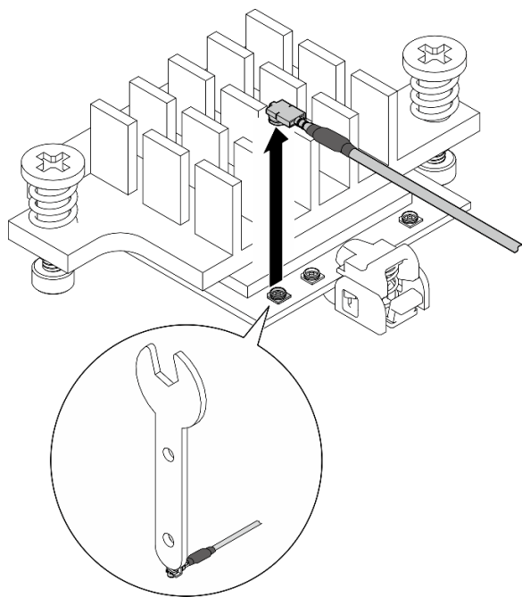
Figura 280. Desconexión del cable
