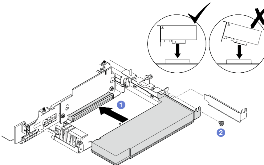
Figura 245. Instalación del adaptador PCIe
