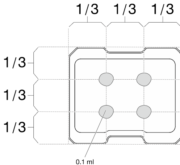
Figura 218. Forma correcta de la grasa térmica
