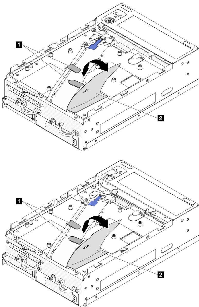
Figura 156. Disposición de los cables de la placa de E/S
