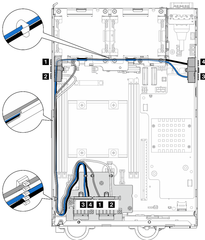
Figura 327. Disposición de los cables para los conjuntos de SMA
