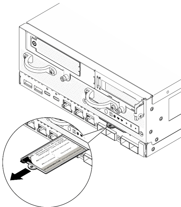
Figura 277. Etiqueta de acceso de red de Lenovo XClarity Controller en la pestaña de información extraíble.
