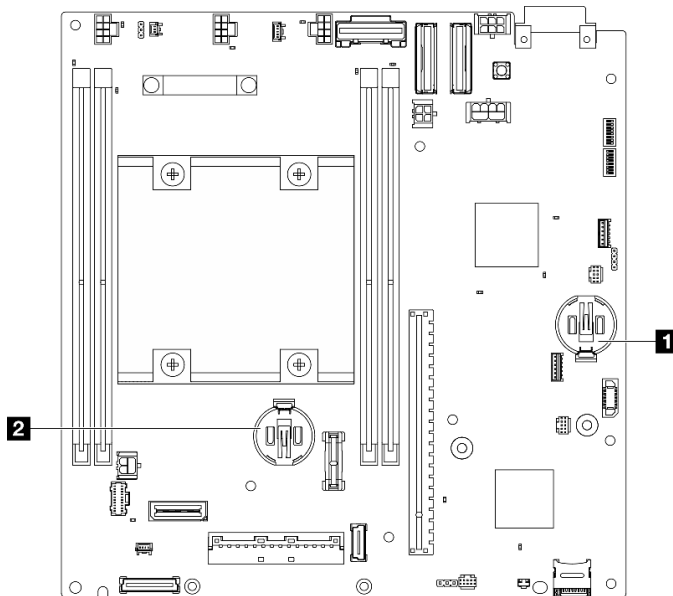
Figura 120. Ubicaciones de la batería de CMOS en la placa del sistema
