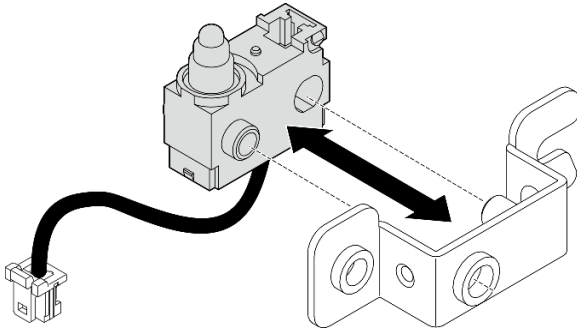
Figura 150. Separación del conmutador de intrusión del soporte
