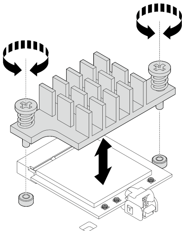
Figura 281. Extracción del disipador de calor del módulo de WLAN/Bluetooth
