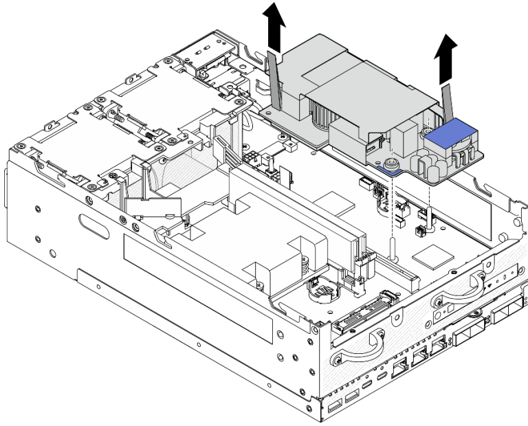
Figura 136. Extracción de la unidad de fuente de alimentación interna
