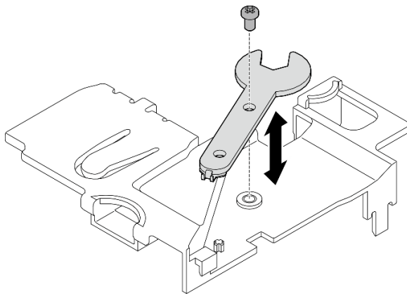
Figura 92. Desenganche de la llave
