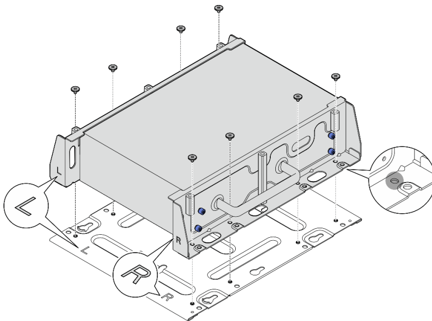
Figura 31. Extracción de la placa inferior
