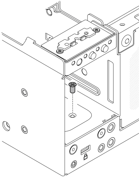
Figura 165. Aflojado del tornillo
