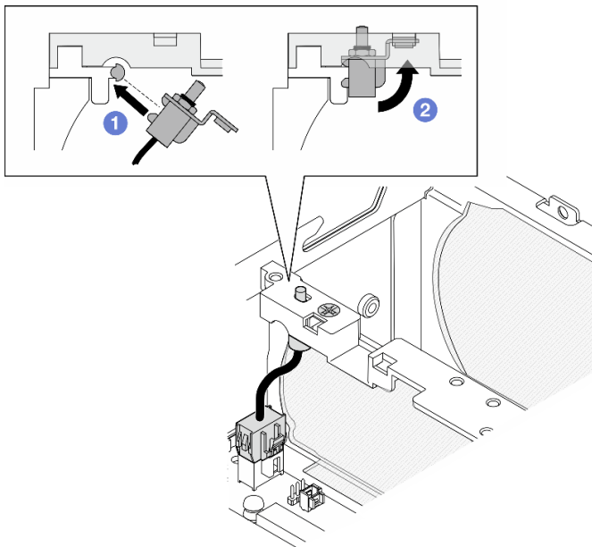
Figura 124. Instalación del conmutador de intrusión con cable
