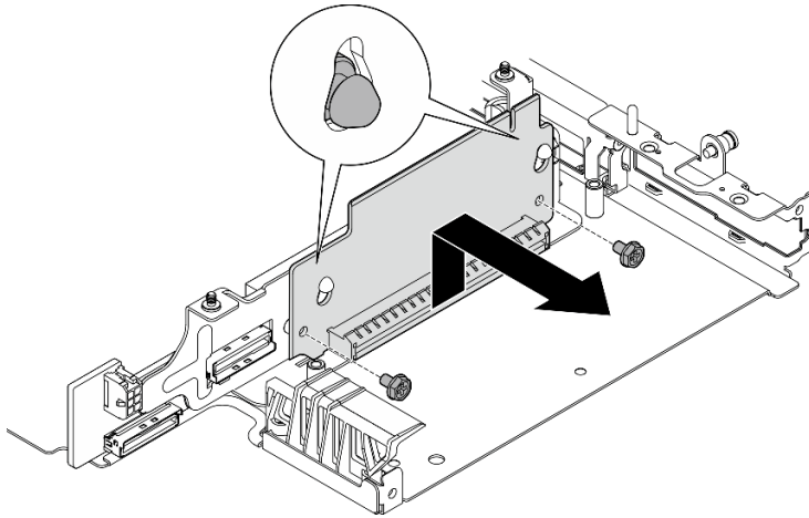
Figura 240. Extracción de la tarjeta de expansión
