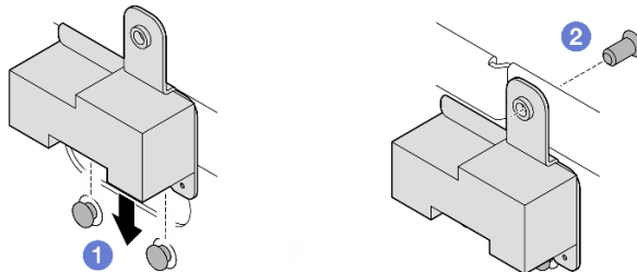
Figura 321. Instalación del relleno de SMA
