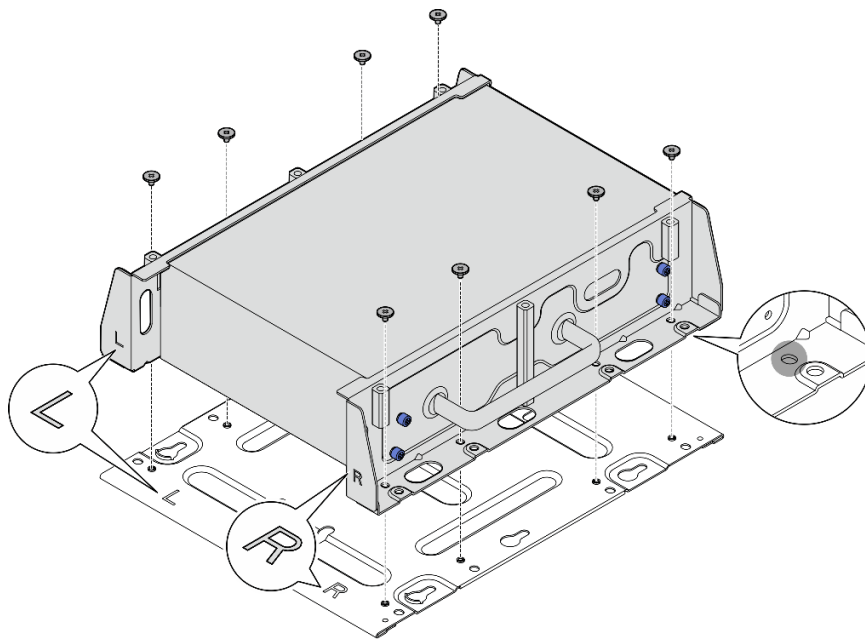
Figura 54. Extracción de la placa inferior
