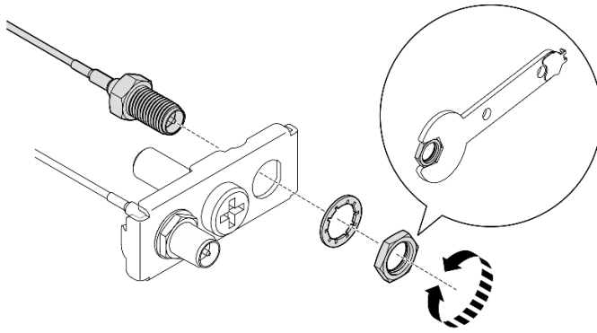
Figura 319. Soltar los cables del soporte
