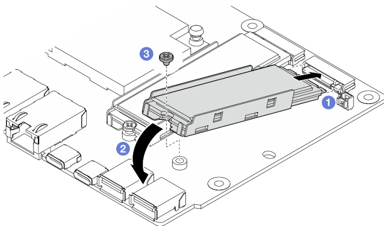
Figura 162. Instalación de una unidad M.2
