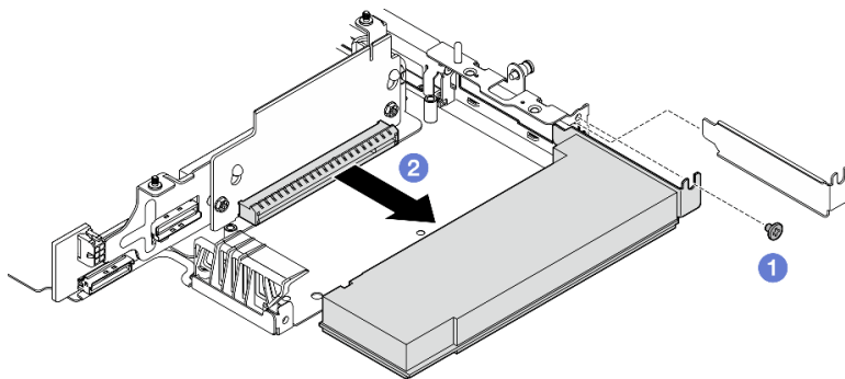
Figura 239. Extracción del adaptador PCIe
