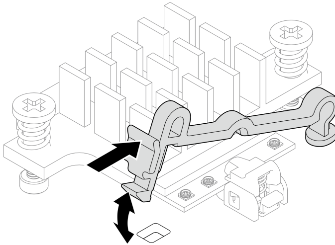
Figura 98. Inserción del soporte de cable
