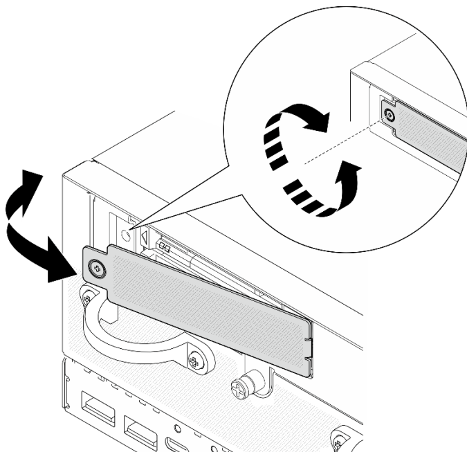
Figura 81. Instalación del marco biselado
