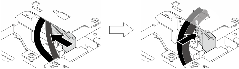
Figura 264. Disposición de los cables
