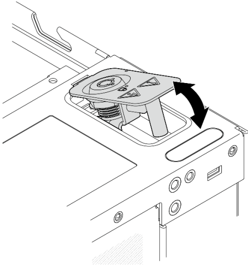
Figura 171. Instalación del bloqueo de seguridad del sistema
