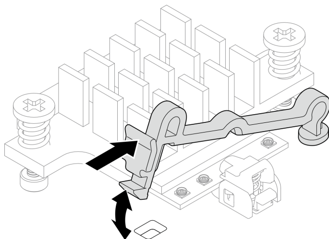
Figura 278. Levantamiento del soporte del cable
