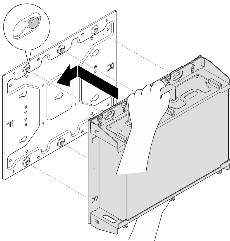
Figura 47. Instalación del soporte del nodo
