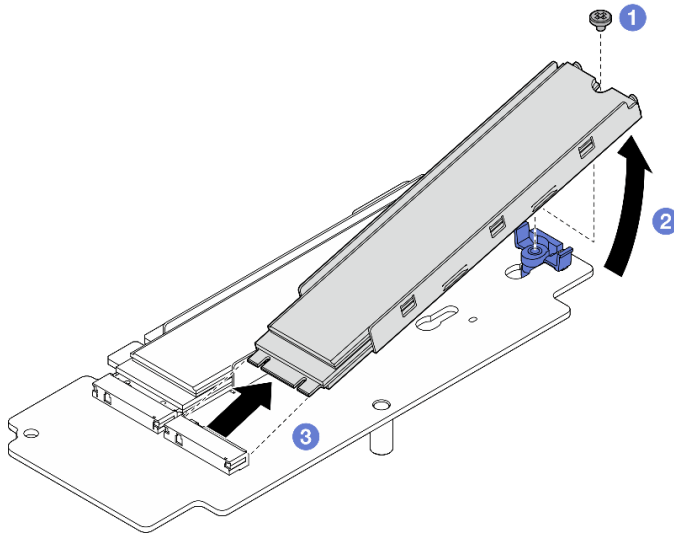
Figura 238. Extracción de una unidad M.2
