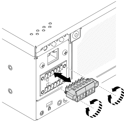
Figura 339. Instalación del cabezal
