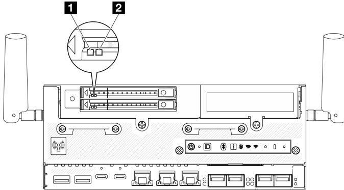
Figura 347. LED de la unidad
