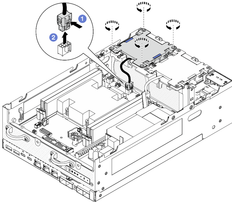
Figura 126. Extracción del módulo de ventilador
