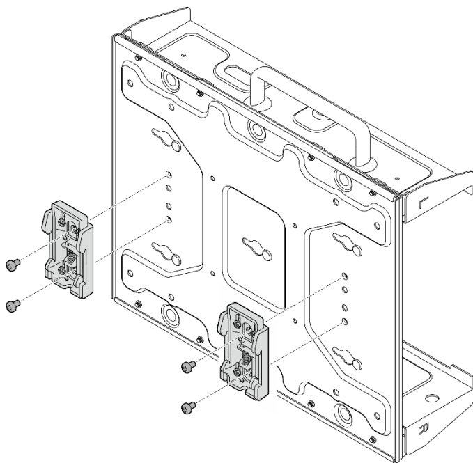
Figura 53. Extracción de los clips del riel DIN
