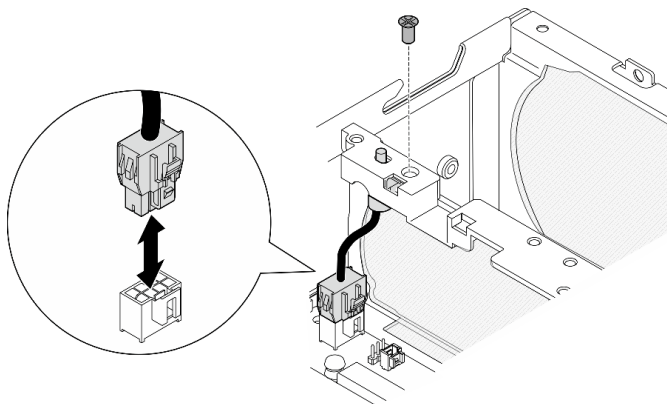
Figura 122. Extracción del conmutador de dirección del ventilador
