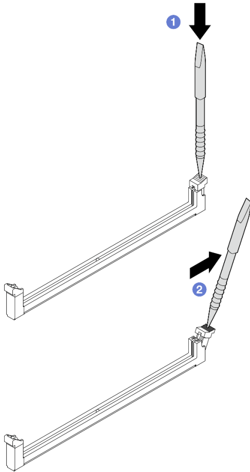
Figura 177. Abrir el seguro de retención
