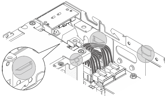
Figura 213. Las ranuras para el deflector de aire de PMB
