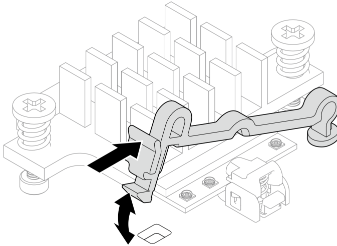
Figura 328. Levantamiento del soporte del cable
