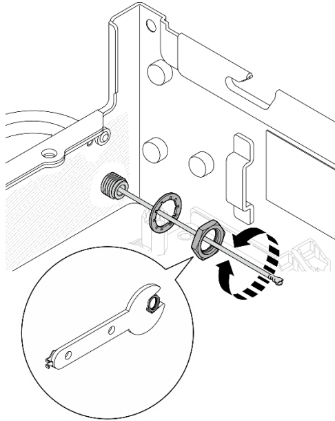
Figura 99. Extracción de la antena Bluetooth
