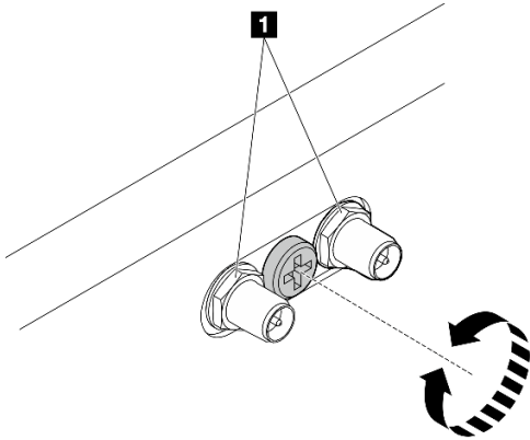
Figura 39. Acortamiento de los conectores SMA
