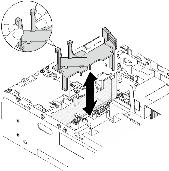
Figura 86. Extracción del deflector de aire
