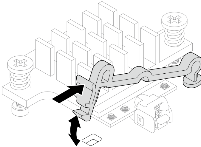
Figura 109. Inserción del soporte de cable
