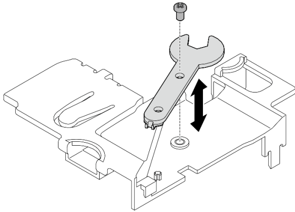
Figura 298. Desenganche de la llave
