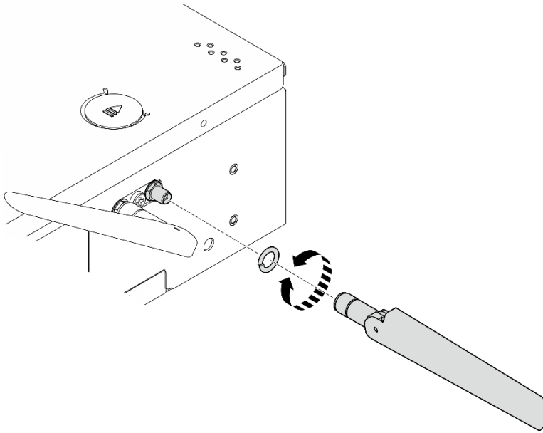
Figura 296. Extracción de una antena WLAN
