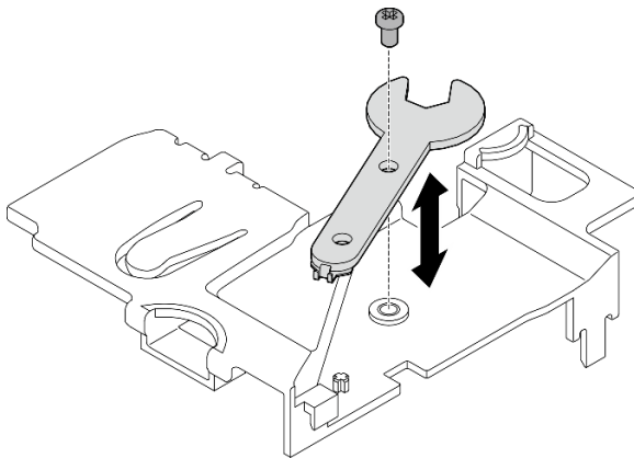
Figura 320. Almacenamiento de la llave
