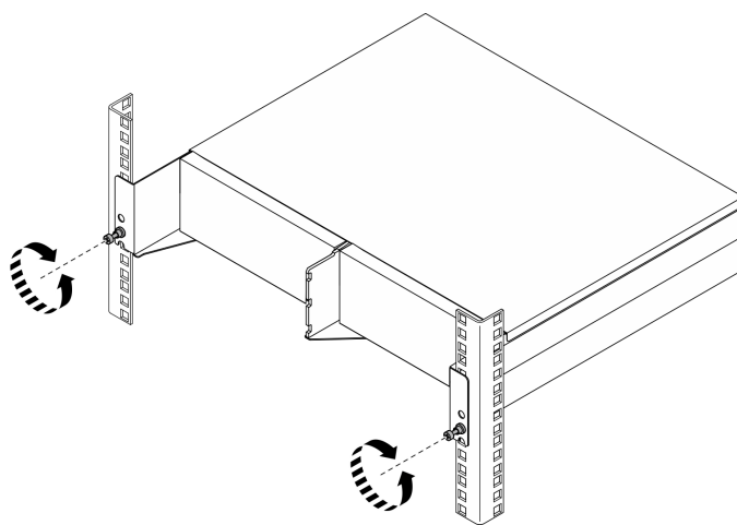
Figura 18. Fijación del alojamiento en el bastidor
