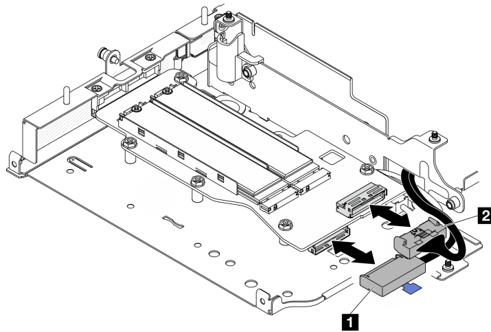
Figura 249. Desconexión del cable de señal
