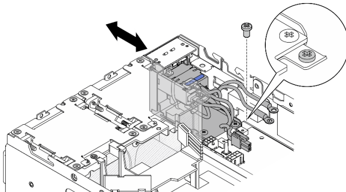
Figura 203. Extracción del módulo PIB de CA
