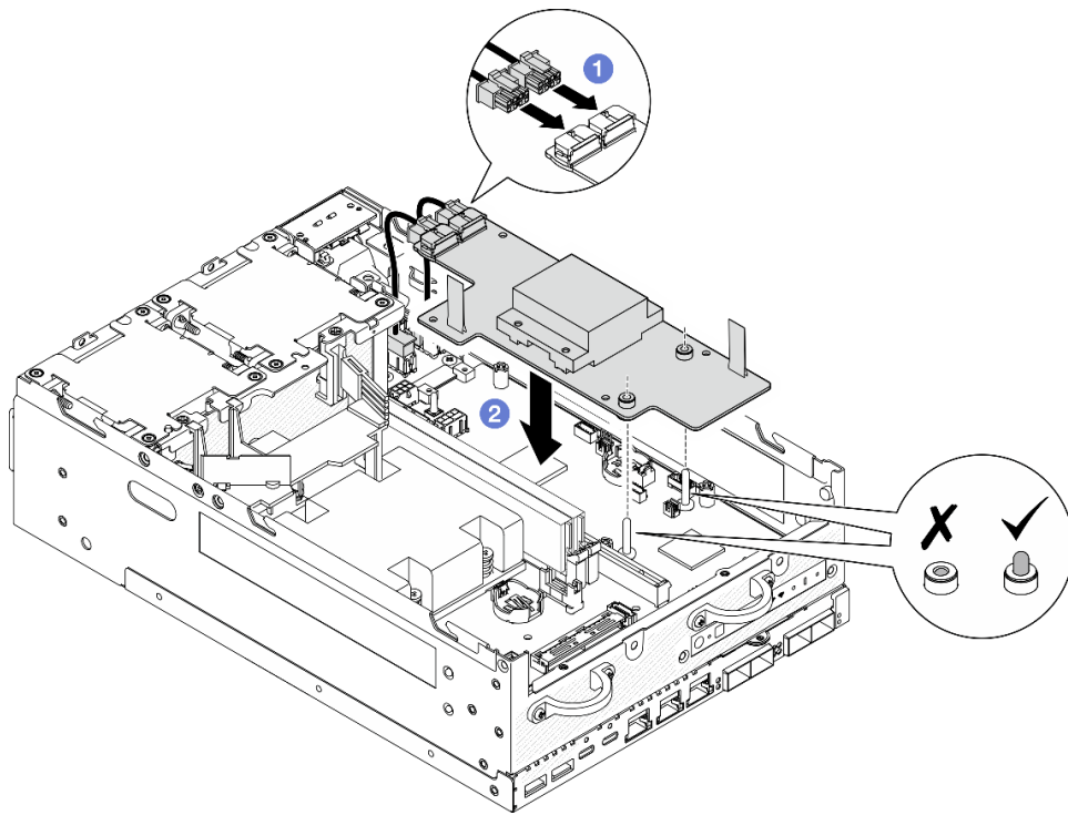
Figura 212. Instalación de la placa del módulo de alimentación
