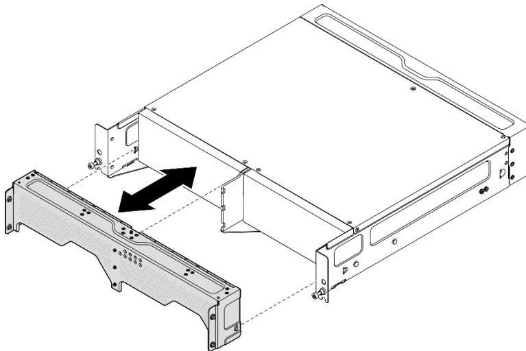
Figura 67. Extracción del soporte de envío
