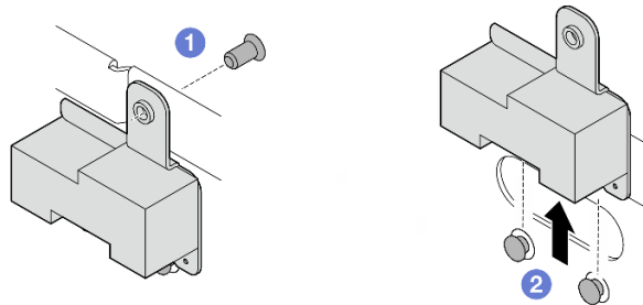
Figura 311. Extracción del relleno de SMA
