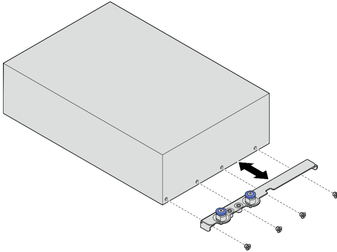
Figura 6. Extracción del soporte del alojamiento
