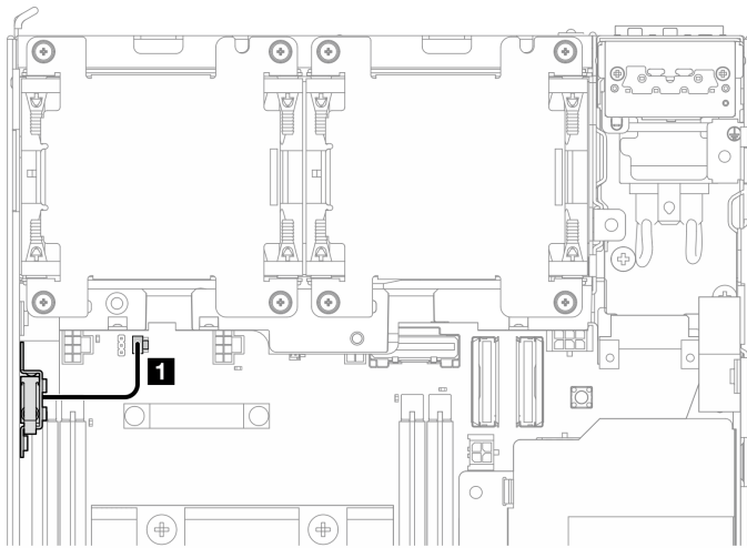
Figura 147. Disposición de los cables del conmutador de intrusión superior
