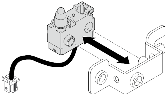
Figura 144. Separación del conmutador de intrusión del soporte
