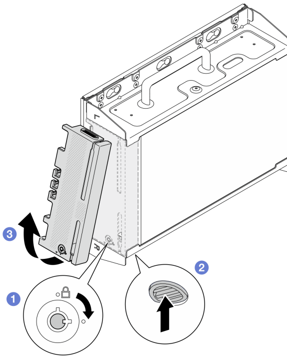
Figura 26. Extracción del marco biselado de seguridad
