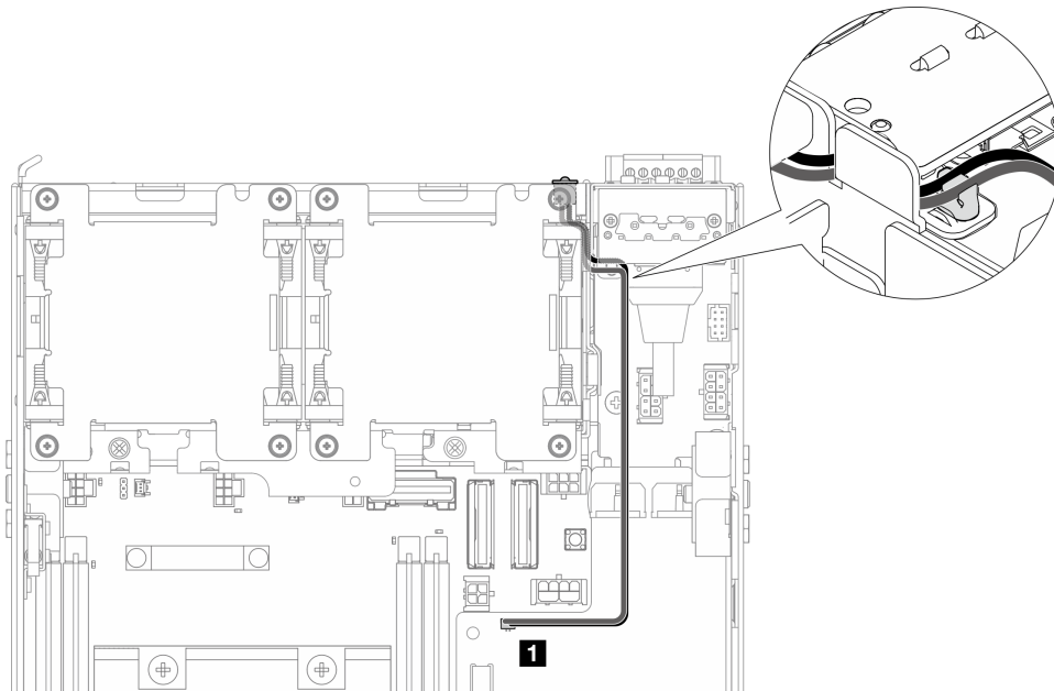
Figura 200. Cable LED de estado de PMB que se conecta a la placa del módulo de alimentación de CC (PMB de CC)
