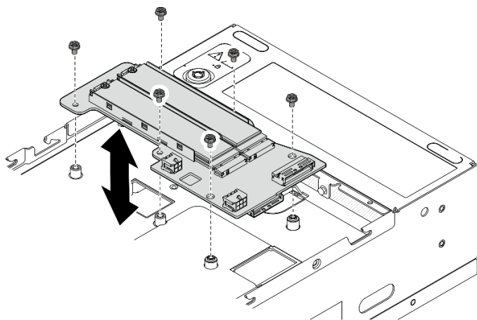
Figura 113. Extracción del adaptador con cable M.2 inferior
