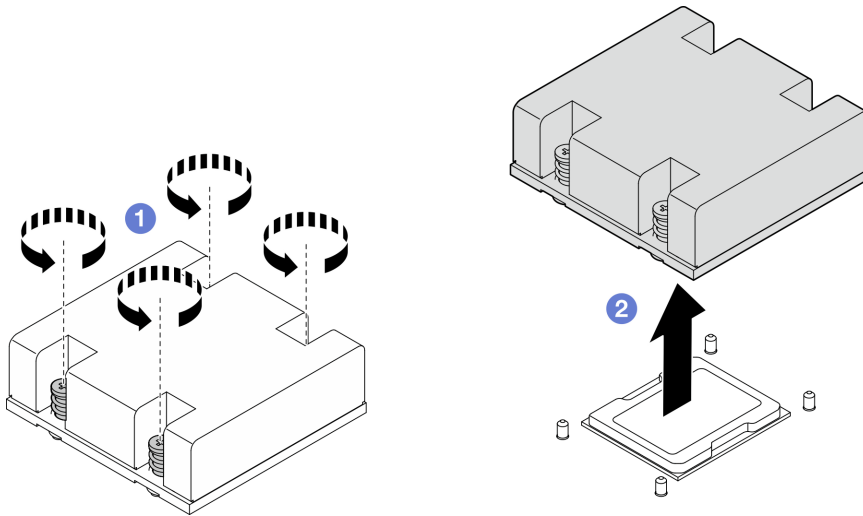
Figura 217. Extracción del dissipador de calor del procesador
