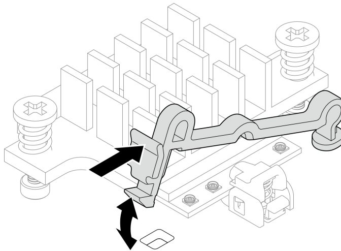
Figura 301. Levantamiento del soporte del cable
