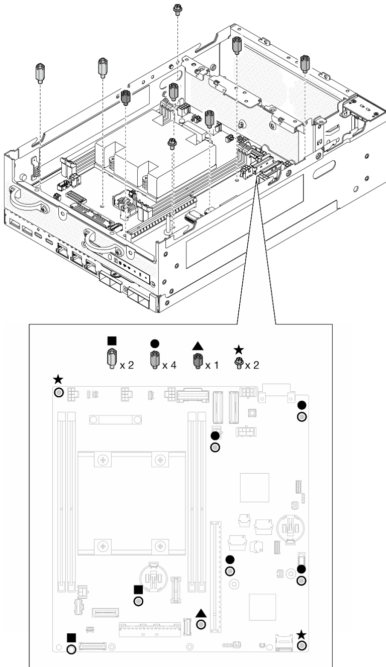
Figura 275. Los tornillos y los separadores de la placa del sistema
