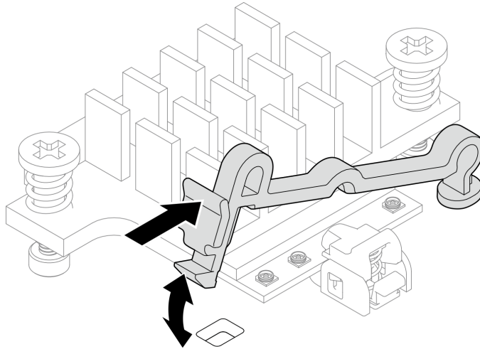
Figura 333. Inserción del soporte de cable
