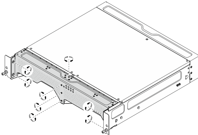
Figura 2. Aflojado de los tornillos
