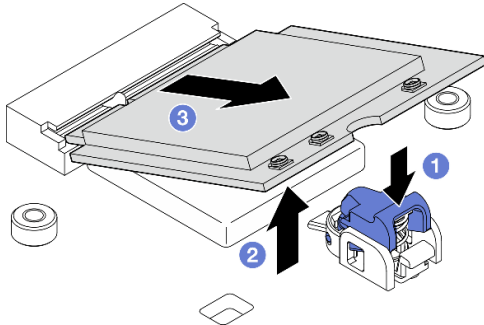
Figura 282. Extracción del módulo de WLAN/Bluetooth
