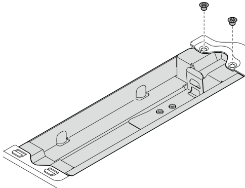
Figura 232. Extracción del compartimiento del módulo de geolocalización
