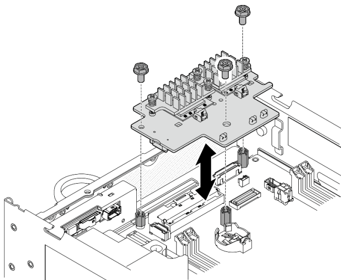
Figura 93. Levantamiento del adaptador inalámbrico
