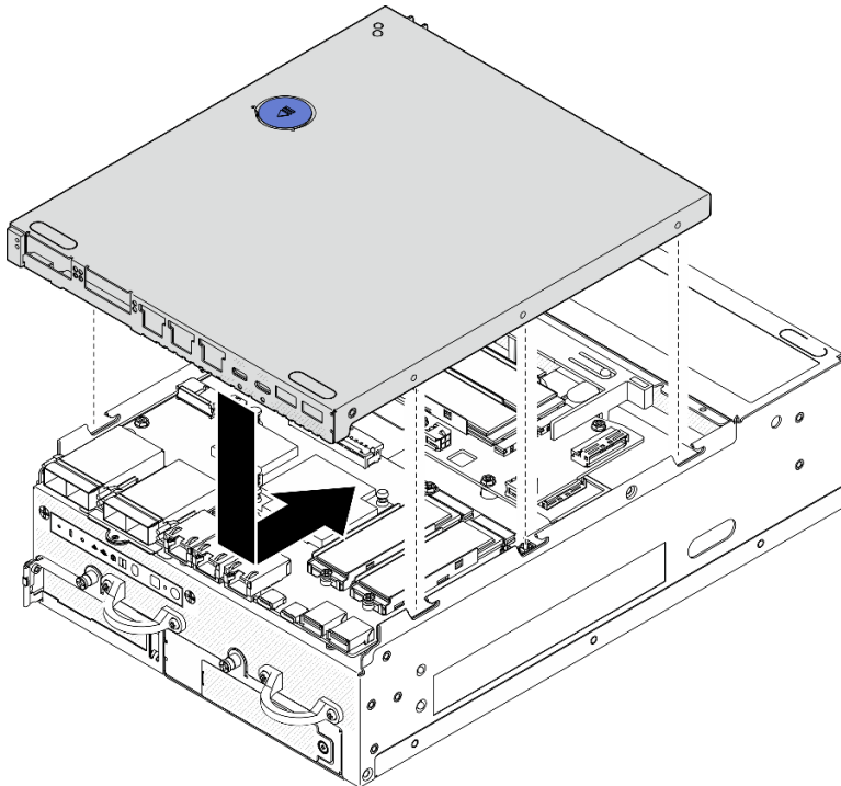
Figura 194. Instalación de la cubierta inferior
