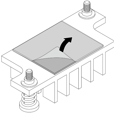
Figura 288. Retirada de la película de la almohadilla térmica
