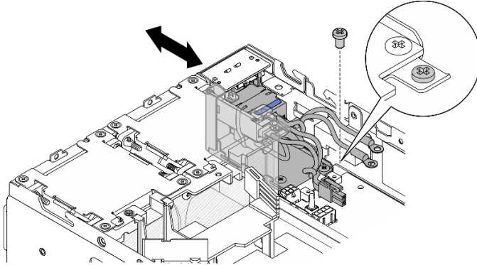
Figura 206. Instalación del módulo PIB
