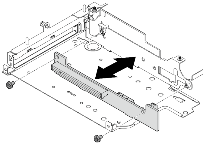
Figura 235. Extracción de la tarjeta de expansión
