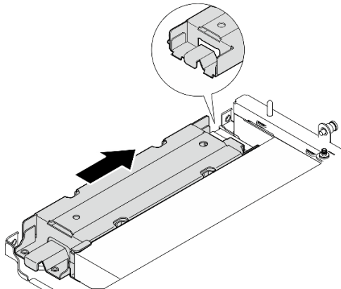
Figura 257. Instalación del compartimiento del módulo de geolocalización
