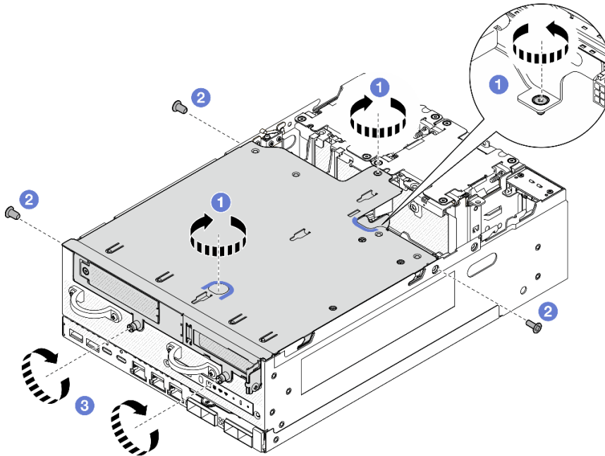
Figura 268. Fijación del conjunto de expansión
