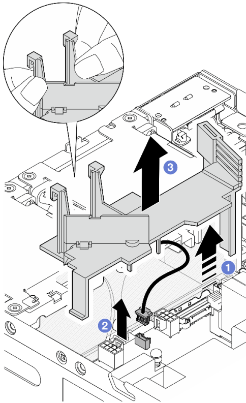
Figura 87. Extracción del deflector de aire
