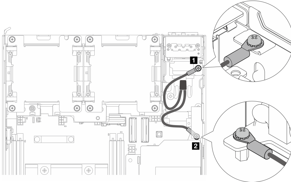
Figura 140. Conectar el cable de tierra
