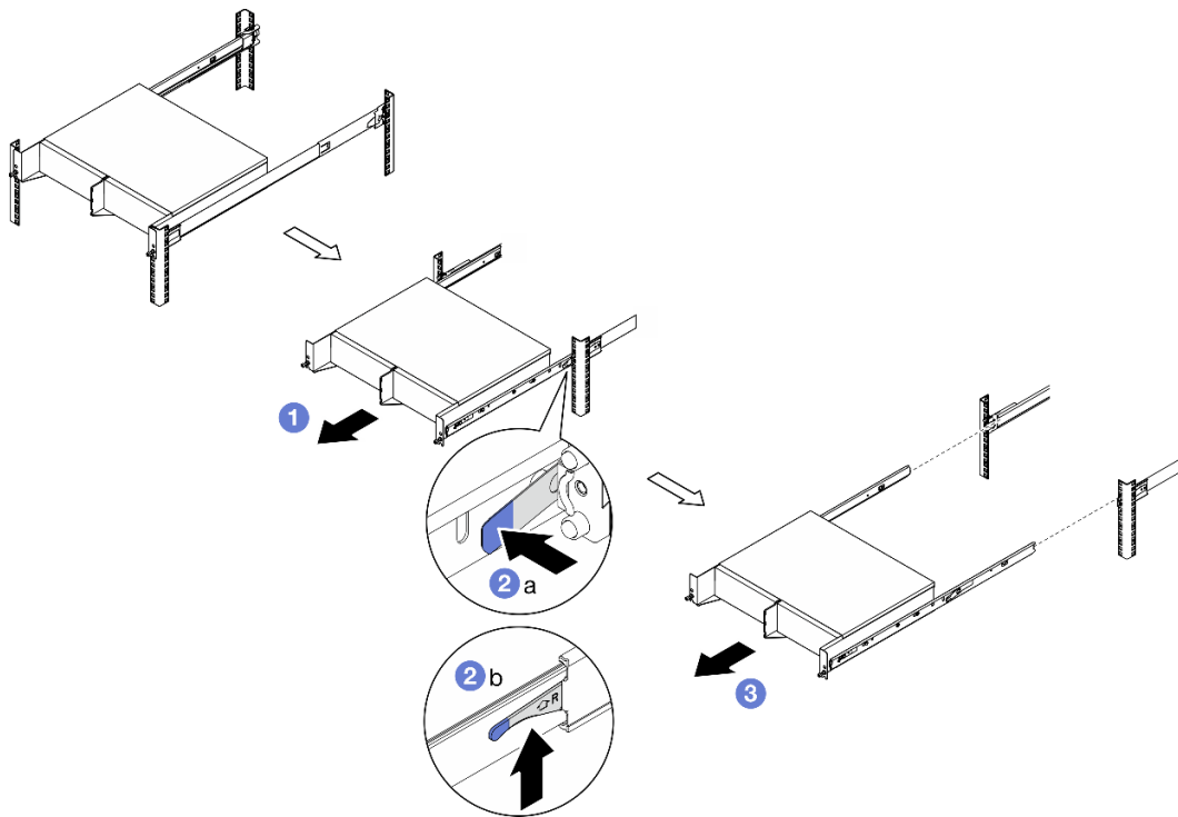
Figura 8. Extracción del alojamiento del bastidor
