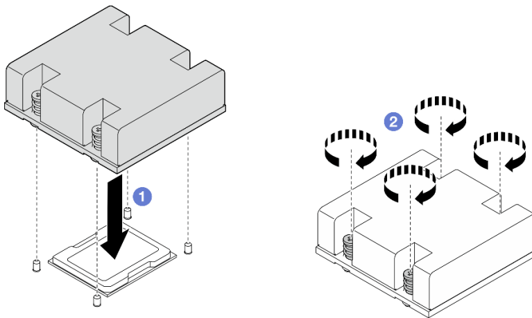
Figura 219. Instalación del disipador de calor del procesador
