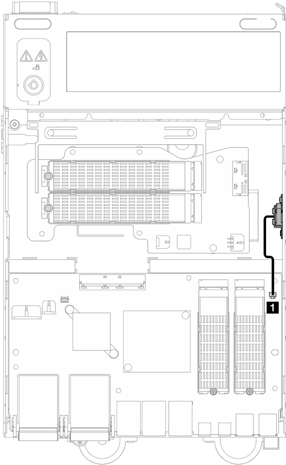
Figura 148. Disposición de los cables del conmutador de intrusión inferior
