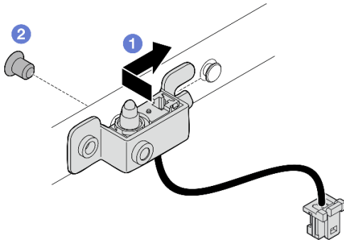
Figura 146. Instalación del conmutador de intrusión con cable
