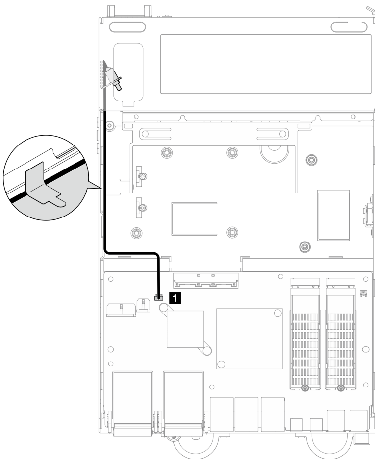
Figura 170. Disposición de los cables del conmutador de posición de bloqueo
