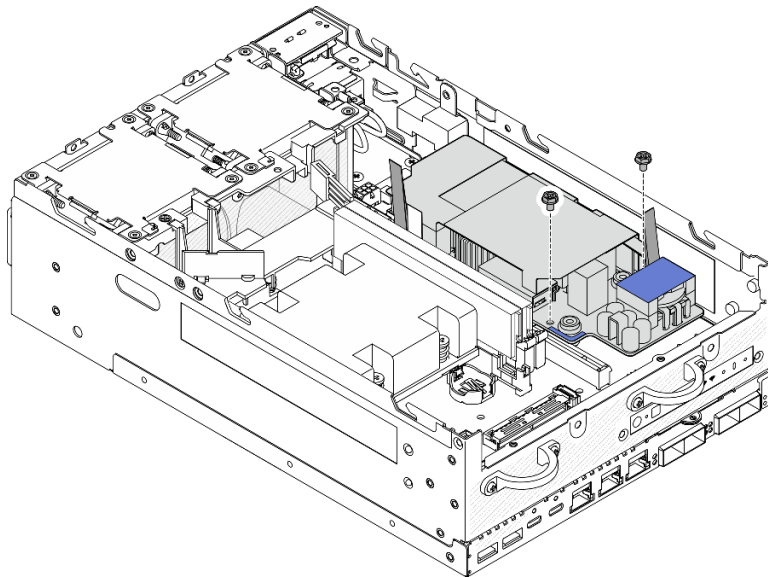
Figura 135. Aflojado de los tornillos
