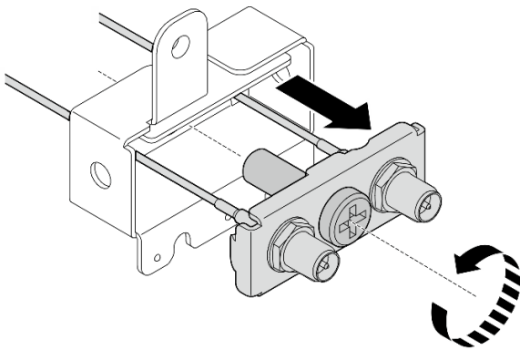
Figura 318. Extracción del soporte
