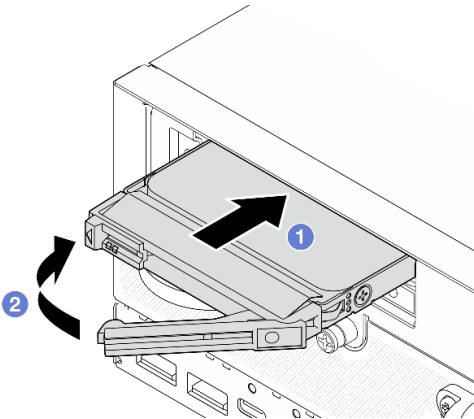
Figura 79. Instalación de una unidad de 7 mm
