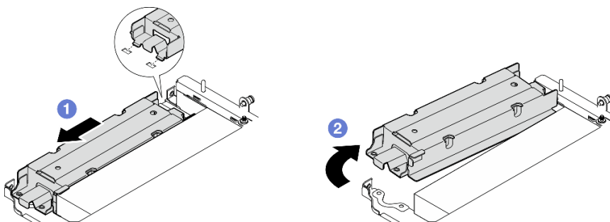
Figura 233. Extracción del compartimiento del módulo de geolocalización
