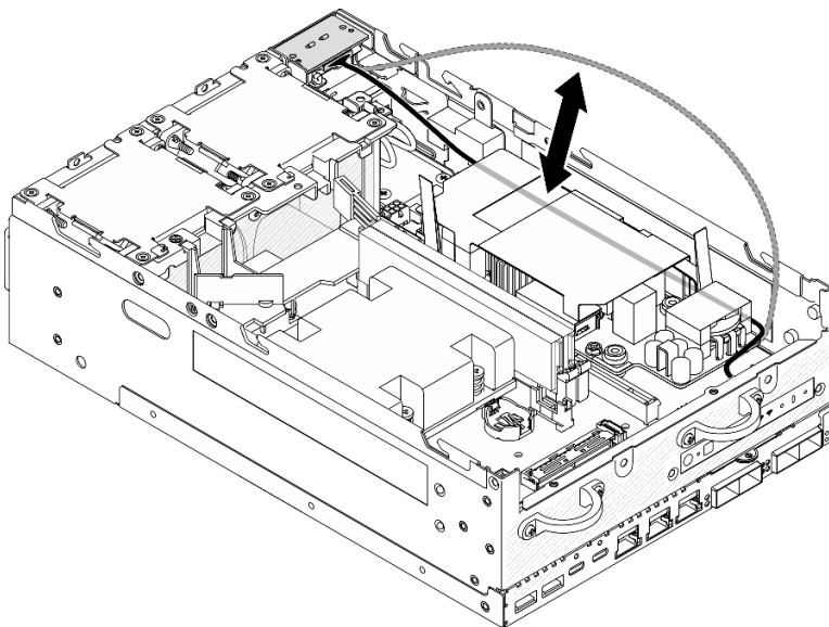
Figura 141. Colocación del cable de señal
