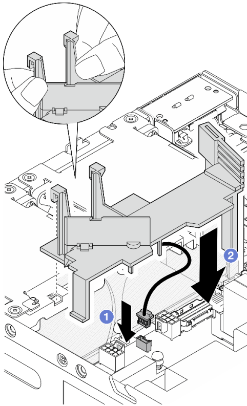
Figura 91. Instalación del deflector de aire
