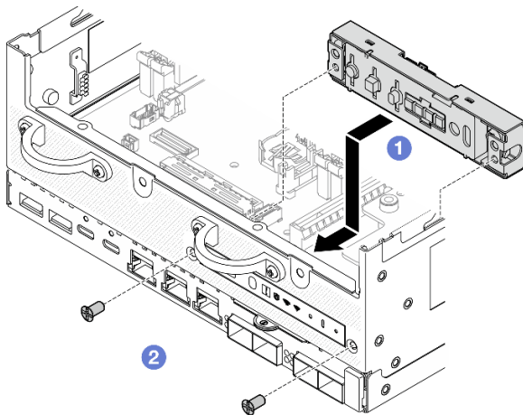
Figura 131. Instalación del panel frontal del operador
