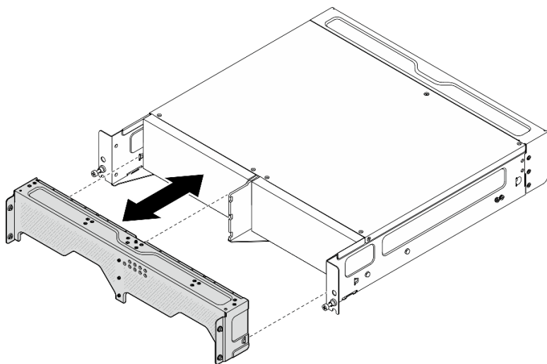
Figura 70. Instalación del soporte de envío
