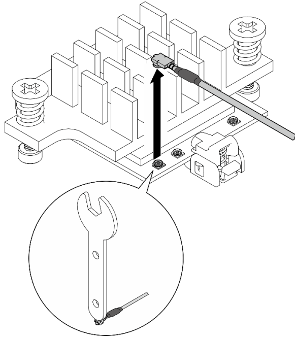
Figura 314. Desconexión del cable
