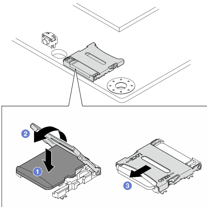
Figura 183. Instalación de la tarjeta MicroSD
