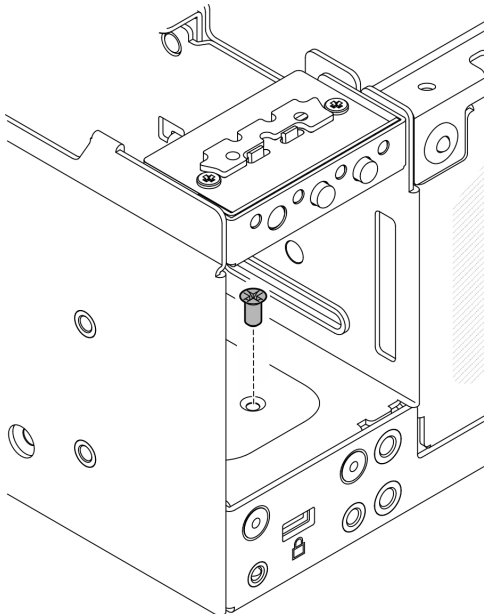
Figura 172. Apriete del tornillo
