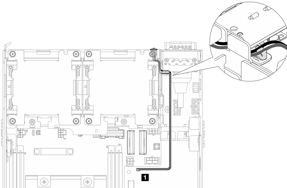
Figura 196. Cable LED de estado de PMB que se conecta a la placa del módulo de alimentación de CC (PMB de CC)
