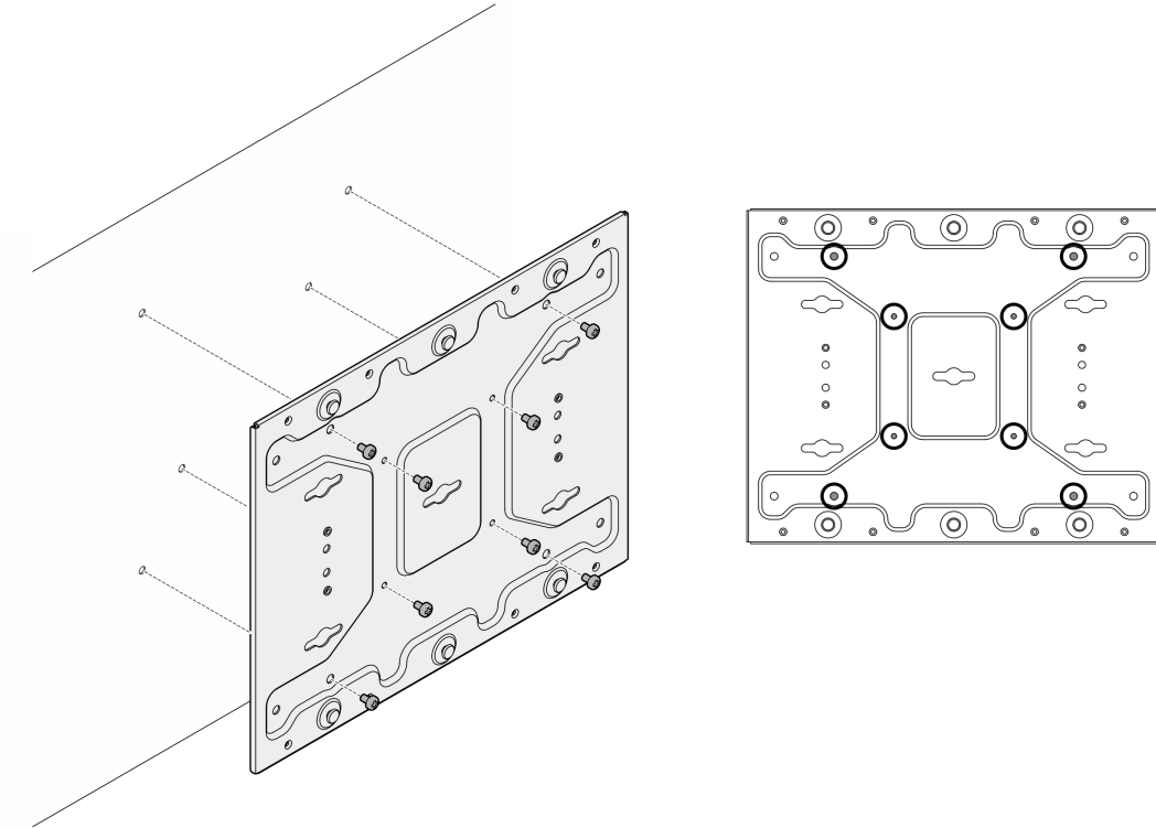
Figura 29. Extracción de la placa de montaje en pared
