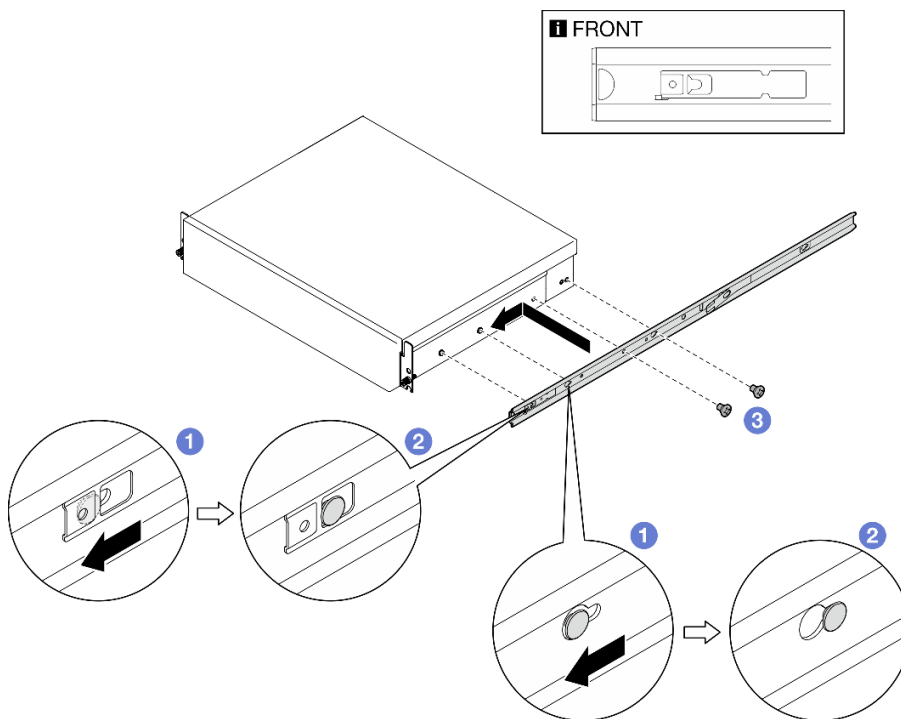
Figura 16. Instalación del riel interno
