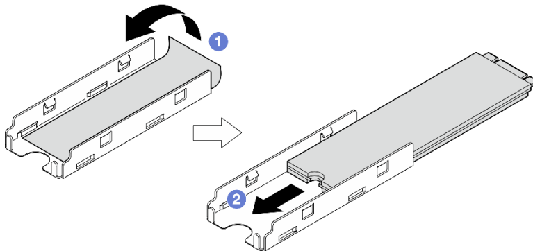
Figura 174. Instalación de la unidad M.2
