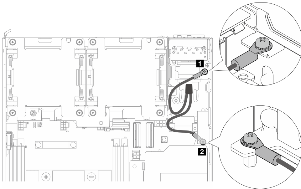
Figura 133. Desconexión de los cables de conexión a tierra
