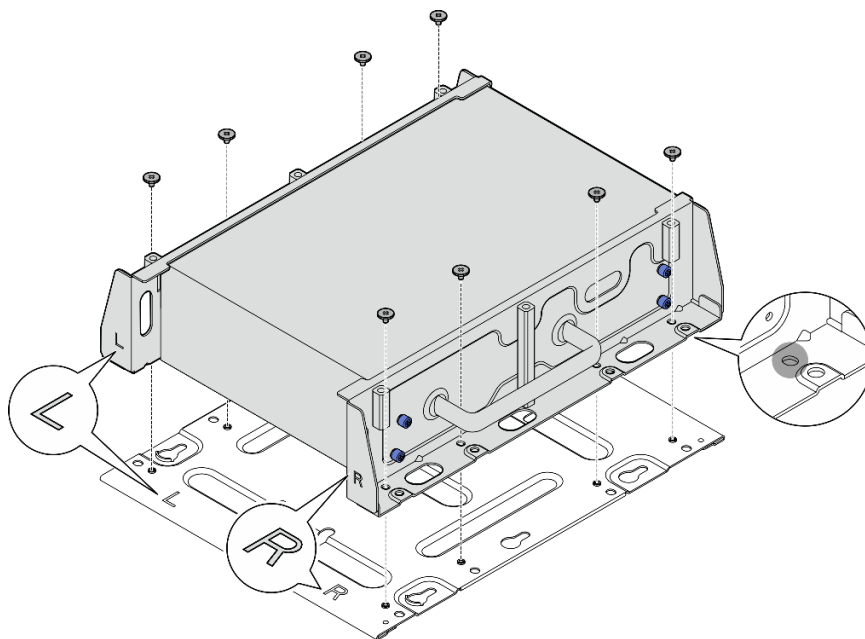
Figura 42. Instalación de la placa inferior
