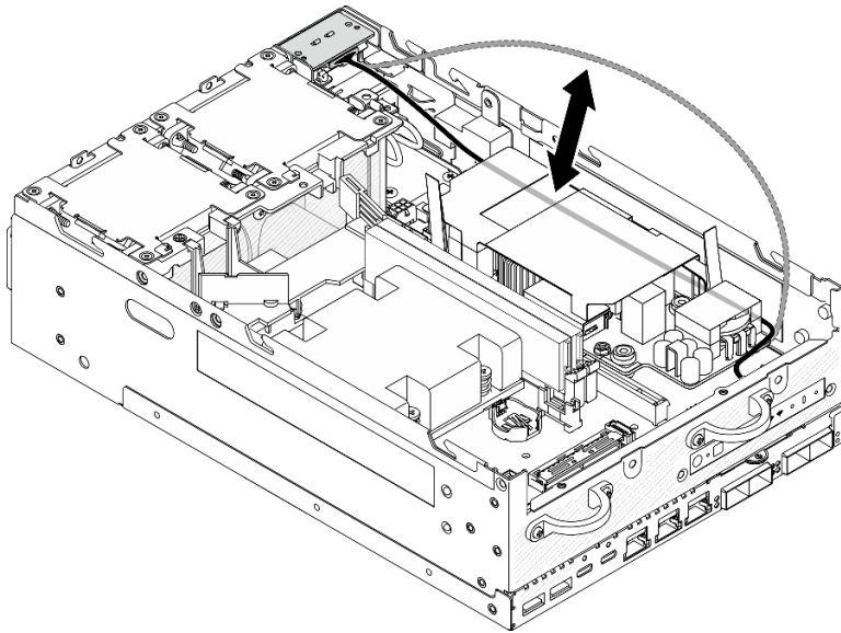
Figura 137. Colocación del cable de señal
