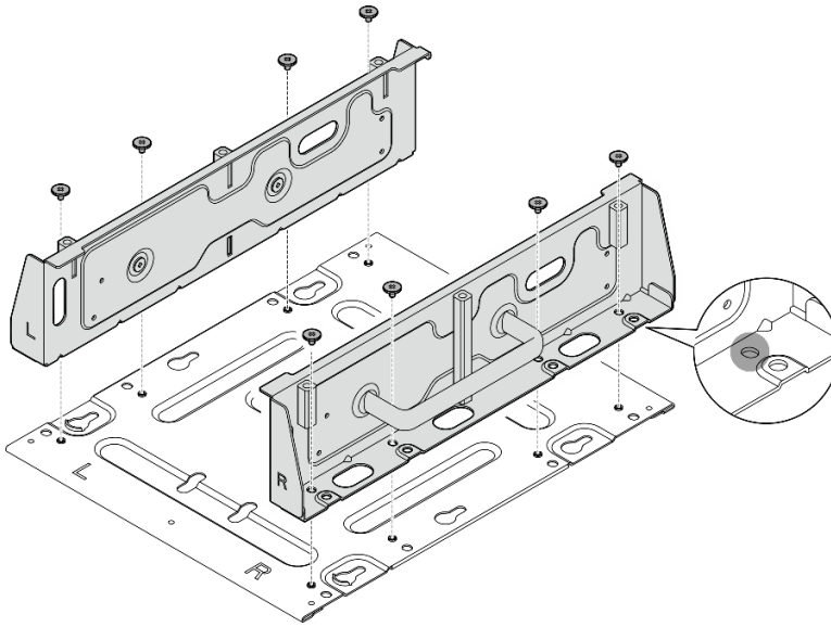
Figura 57. Ensamblaje de la manga del nodo
