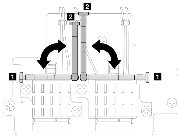
Figura 279. Giro del soporte del cable
