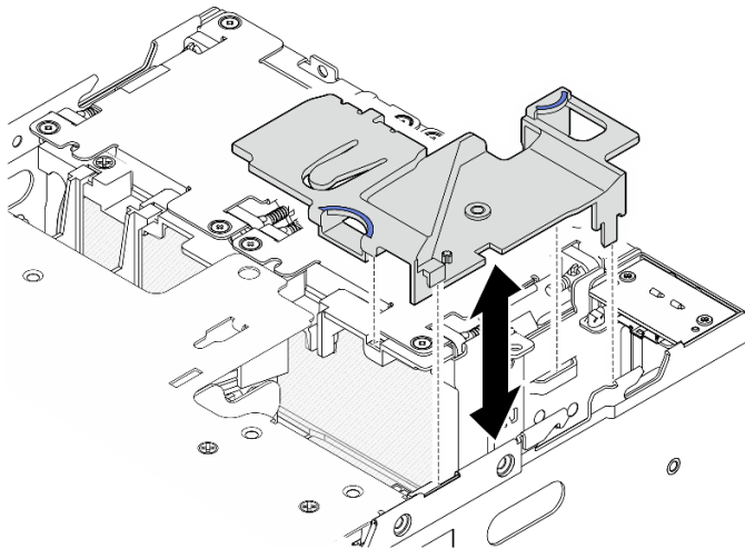
Figura 85. Instalación del deflector de aire
