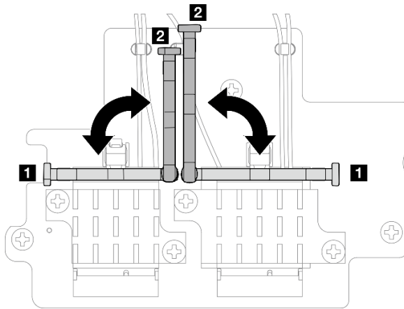
Figura 315. Giro del soporte del cable
