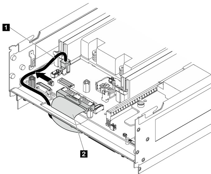
Figura 158. Disposición de los cables de la placa de E/S
