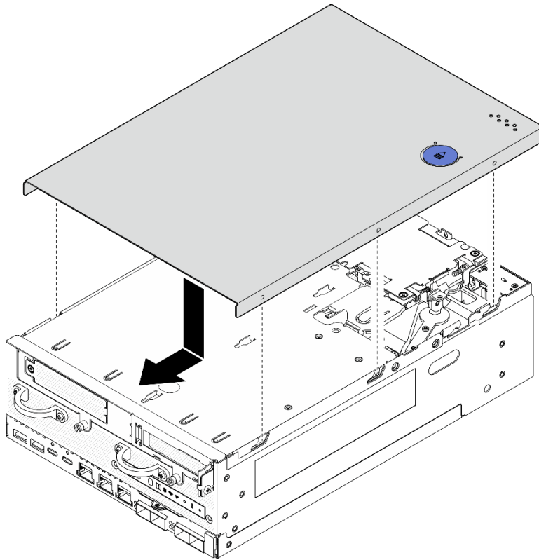
Figura 188. Instalación de la cubierta superior
