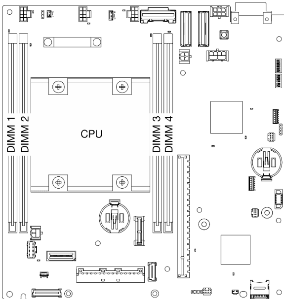
Figura 176. Diseño de los módulos de memoria y el procesador
