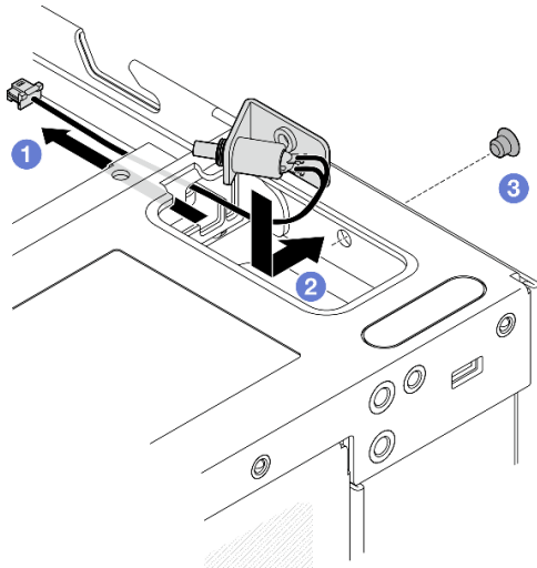
Figura 169. Instalación del conmutador de posición de bloqueo con cable
