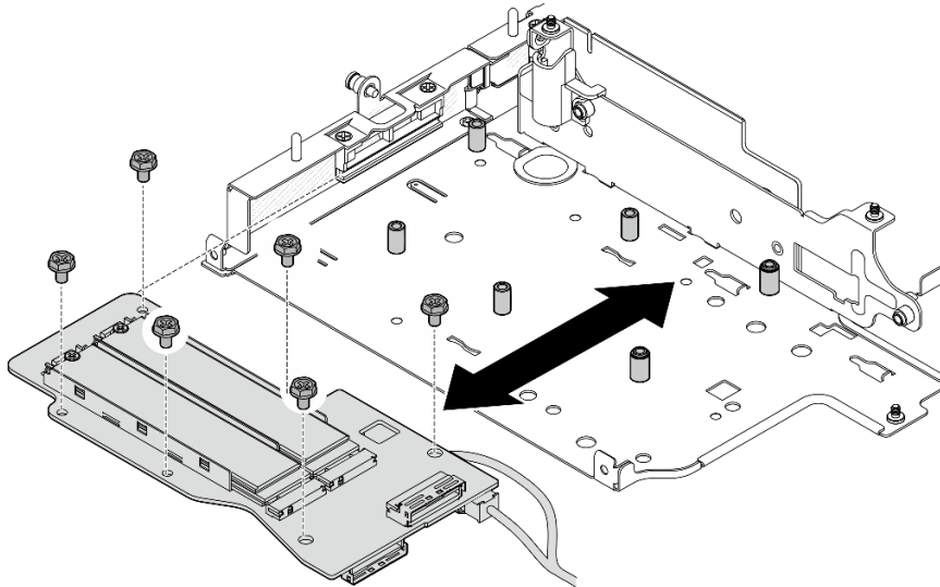
Figura 225. Extracción del adaptador con cable M.2
