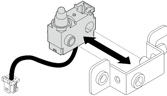
Figura 145. Inserción del conmutador de intrusión en el soporte
