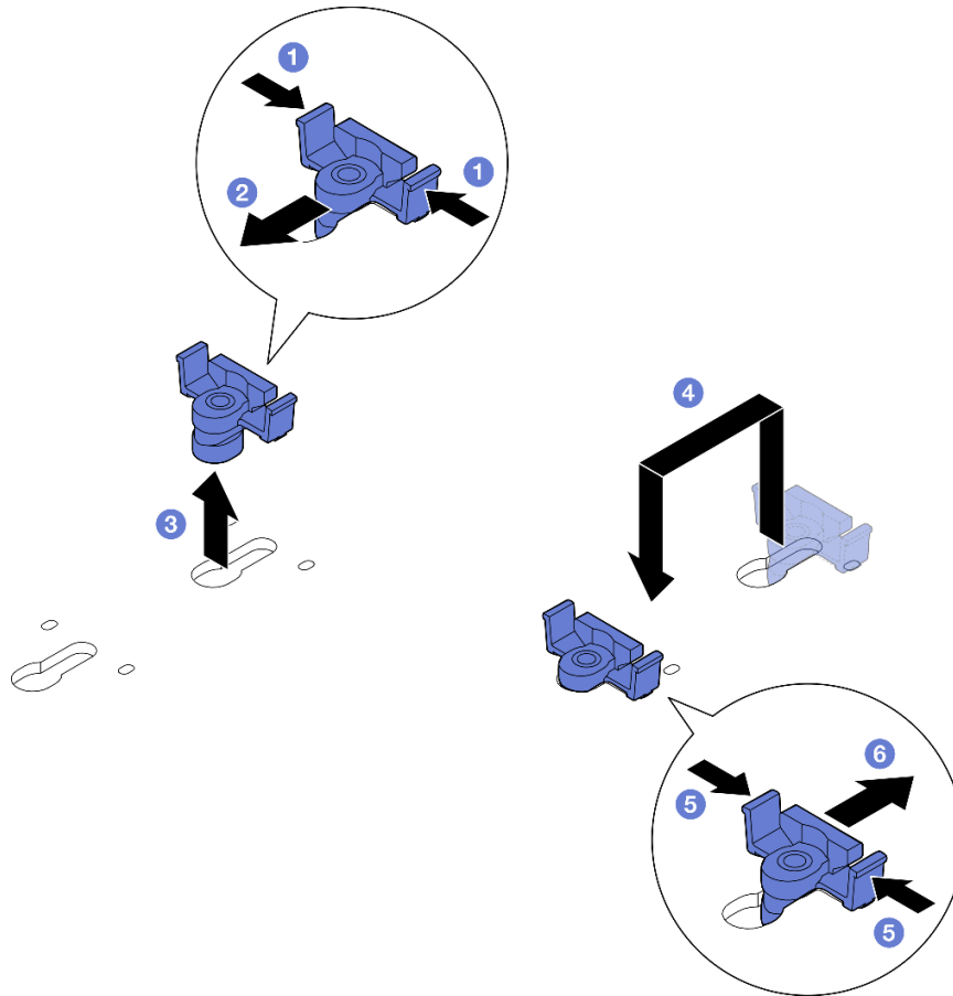
Figura 114. Ajuste del elemento de sujeción M.2
