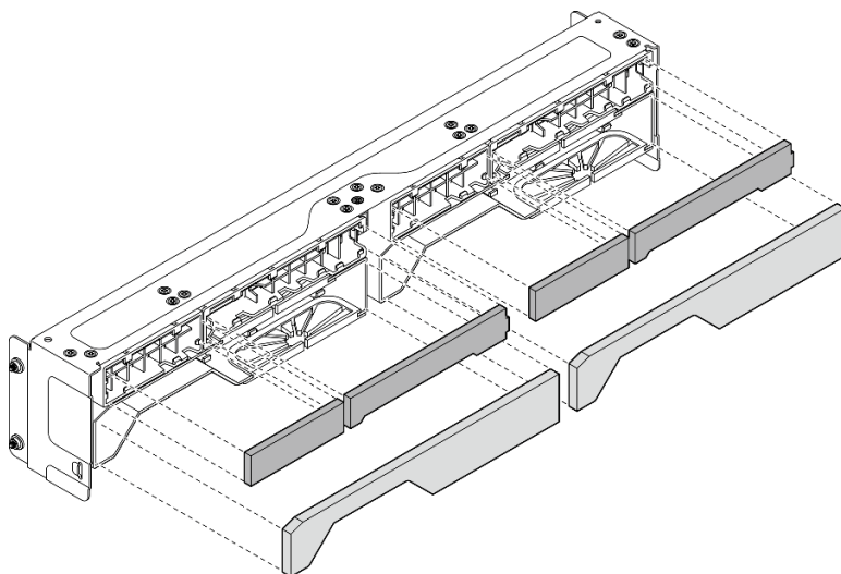
Figura 68. Extracción de los filtro de polvo
