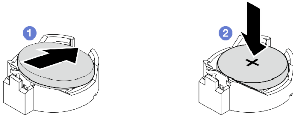
Figura 121. Instalación de la batería CMOS
