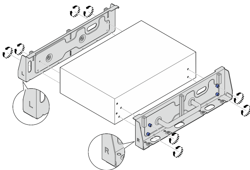
Figura 56. Aflojado de los tornillos ajustables para extraer los soportes laterales
