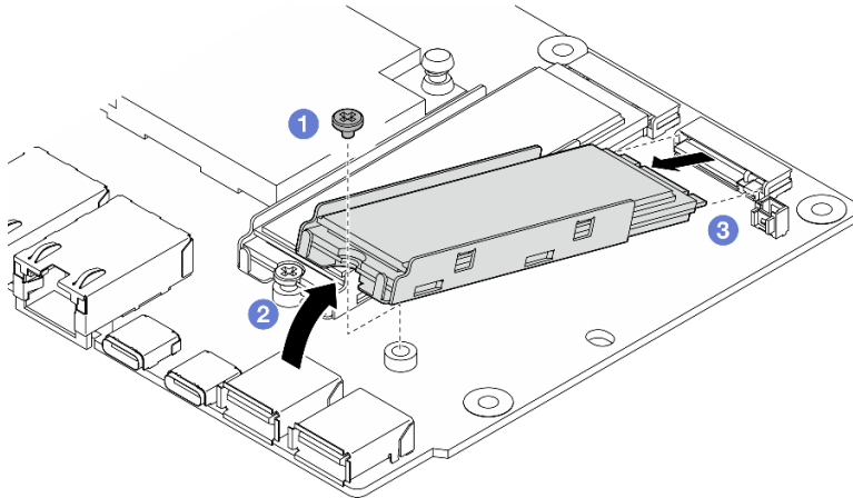
Figura 154. Extracción de una unidad M.2
