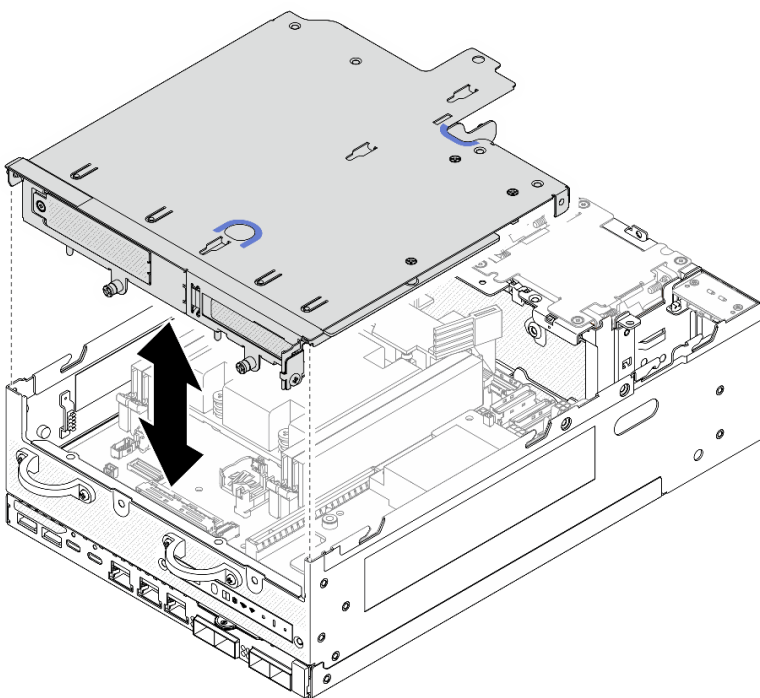
Figura 260. Bajada del conjunto de expansión
