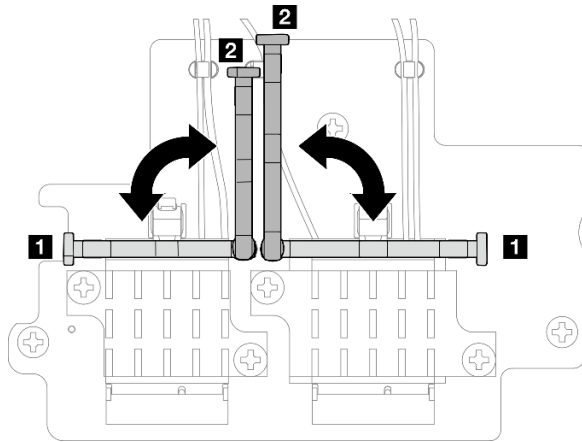
Figura 95. Giro del soporte del cable
