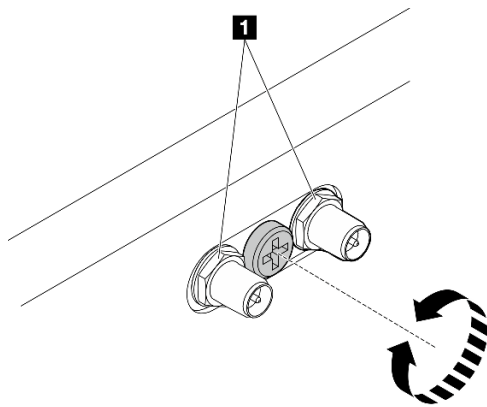
Figura 52. Acortamiento de los conectores SMA
