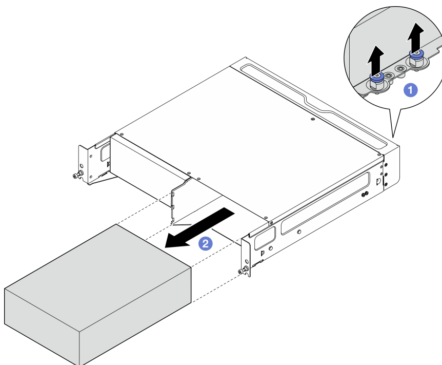
Figura 4. Extracción del nodo
