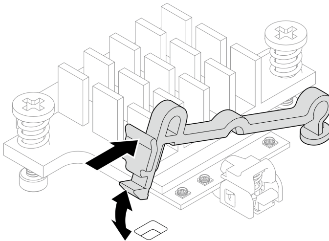
Figura 105. Levantamiento del soporte del cable
