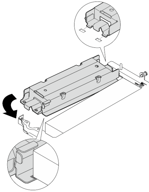
Figura 256. Instalación del compartimiento del módulo de geolocalización
