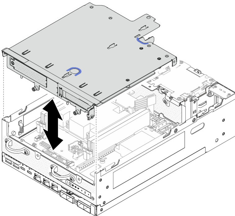
Figura 266. Bajada del conjunto de expansión
