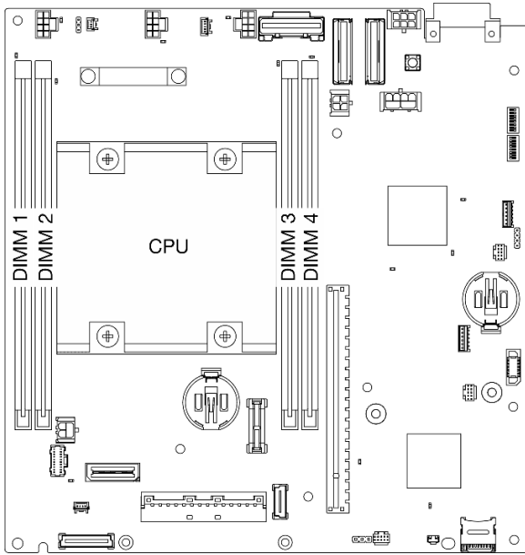
Figura 179. Diseño de los módulos de memoria y el procesador
