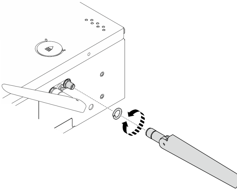
Figura 338. Instalación de una antena WLAN
