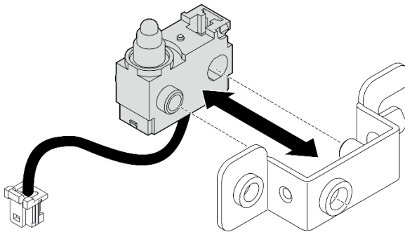
Figura 151. Inserción del conmutador de intrusión en el soporte
