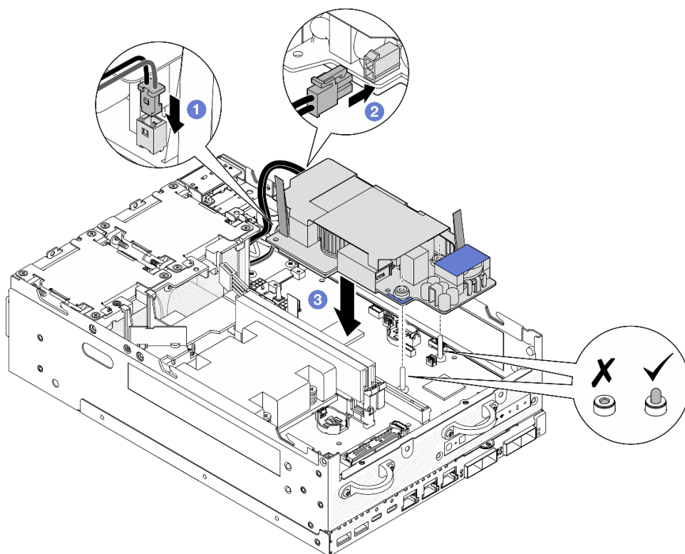
Figura 138. Instalación de la unidad de fuente de alimentación interna
