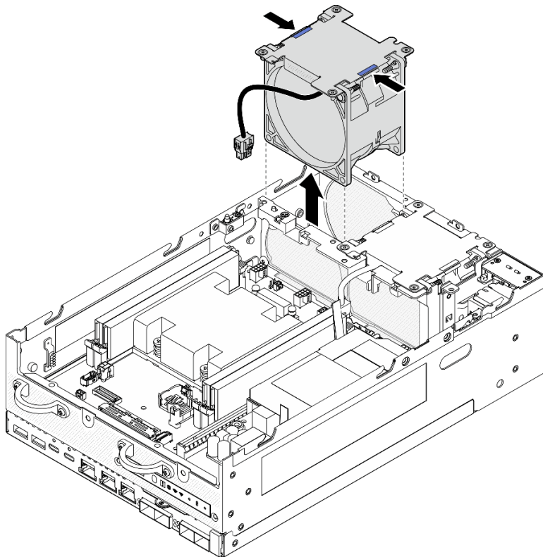
Figura 127. Extracción del módulo de ventilador
