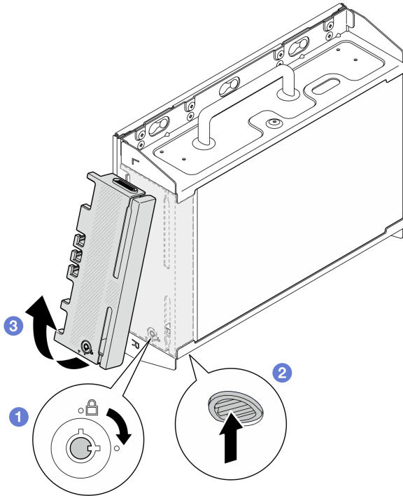
Figura 50. Extracción del marco biselado de seguridad
