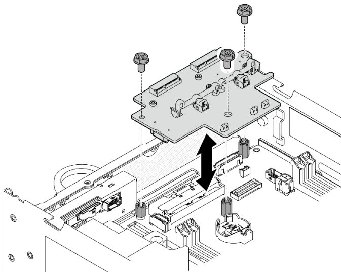
Figura 110. Instalación del adaptador inalámbrico
