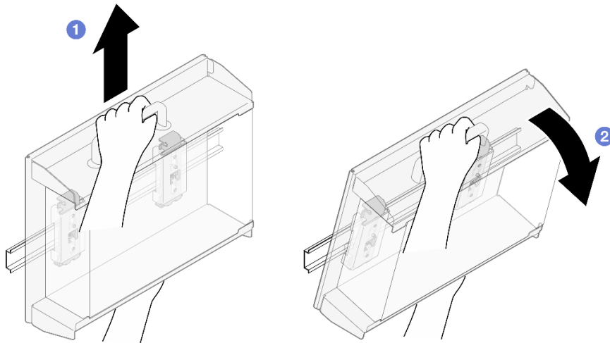
Figura 51. Extracción de la manga del nodo
