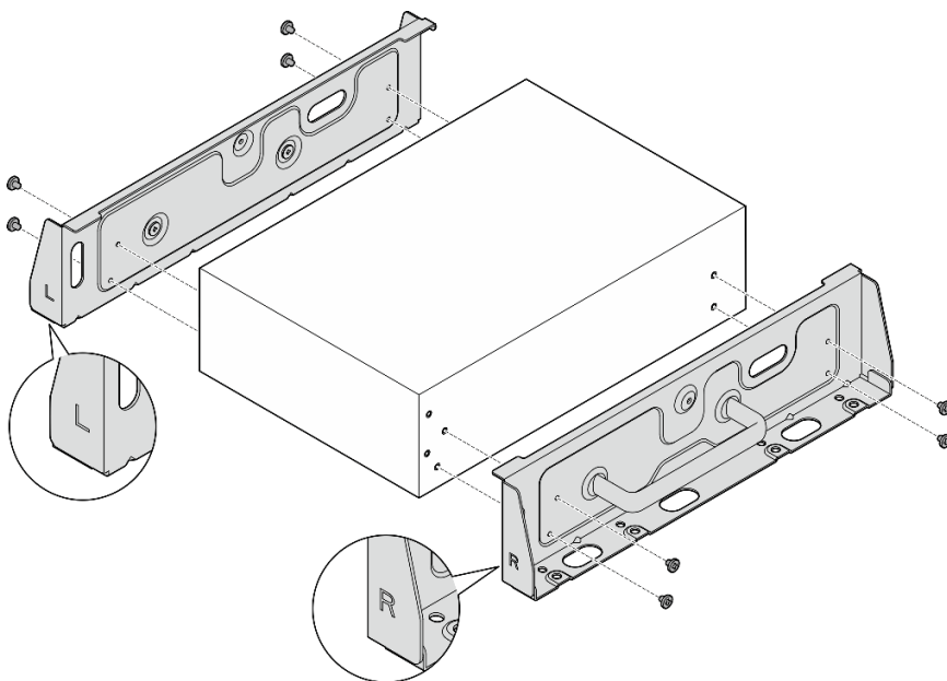
Figura 55. Aflojado de los tornillos para extraer los soportes laterales
