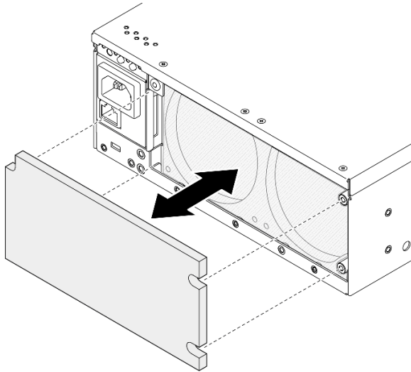
Figura 73. Extracción del filtro de polvo
