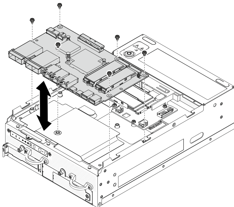
Figura 155. Extracción de la placa del módulo de E/S
