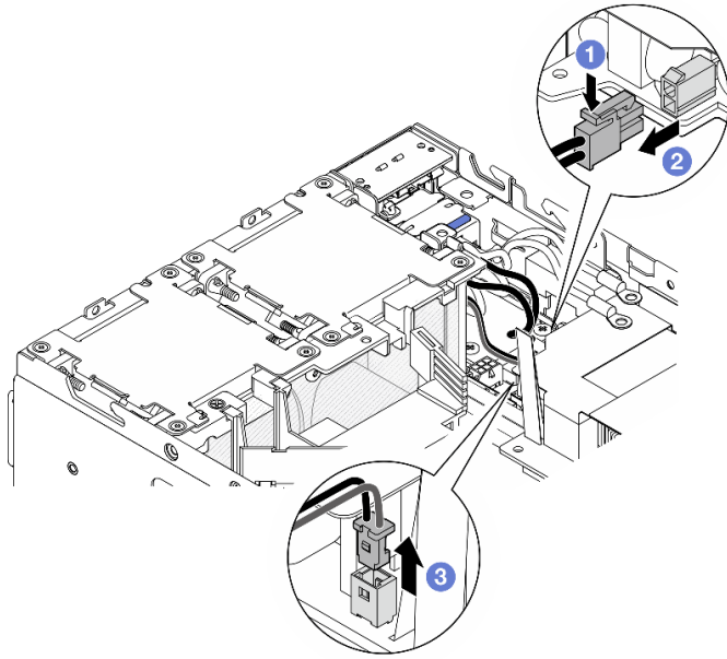
Figura 134. Desconexión de los cables
