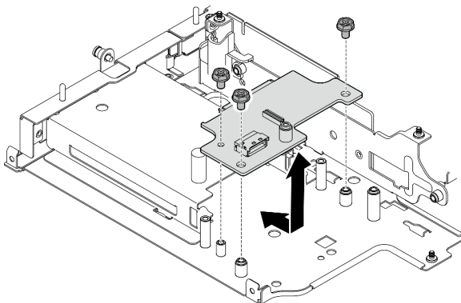
Figura 252. Instalación de la placa posterior 1
