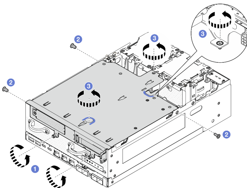
Figura 222. Desenganche del conjunto de expansión
