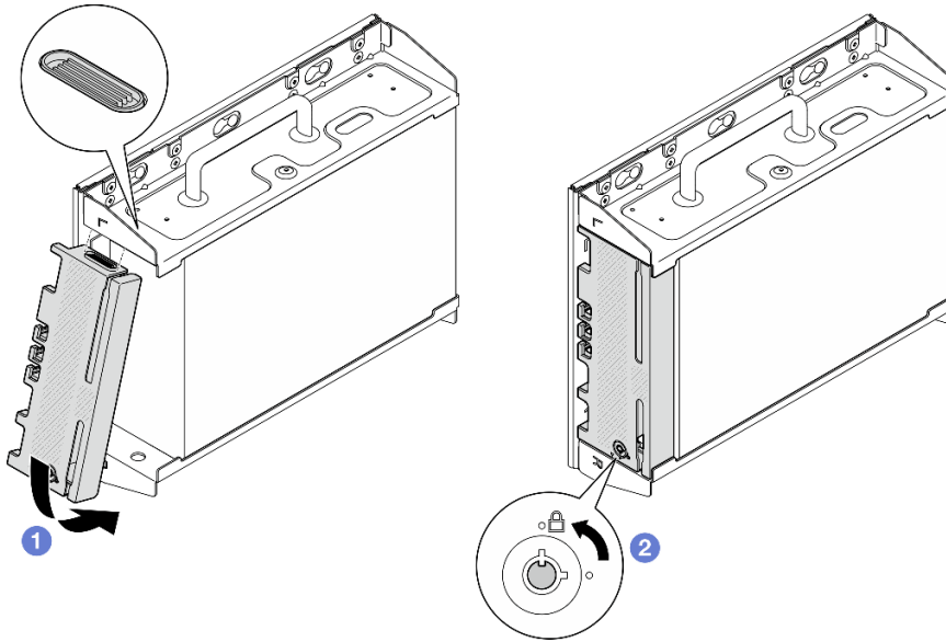
Figura 65. Instalación del marco biselado de seguridad
