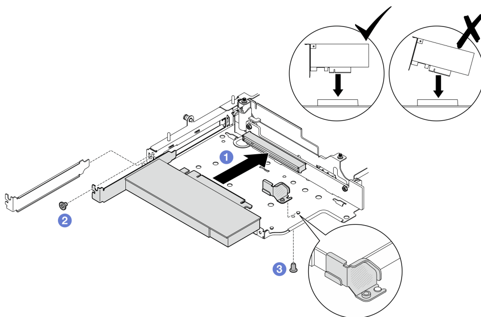
Figura 251. Instalación del adaptador PCIe
