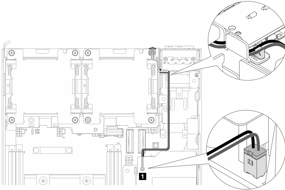
Figura 201. Cable LED de estado de PMB que se conecta a la unidad de fuente de alimentación interna (PMB de CA)
