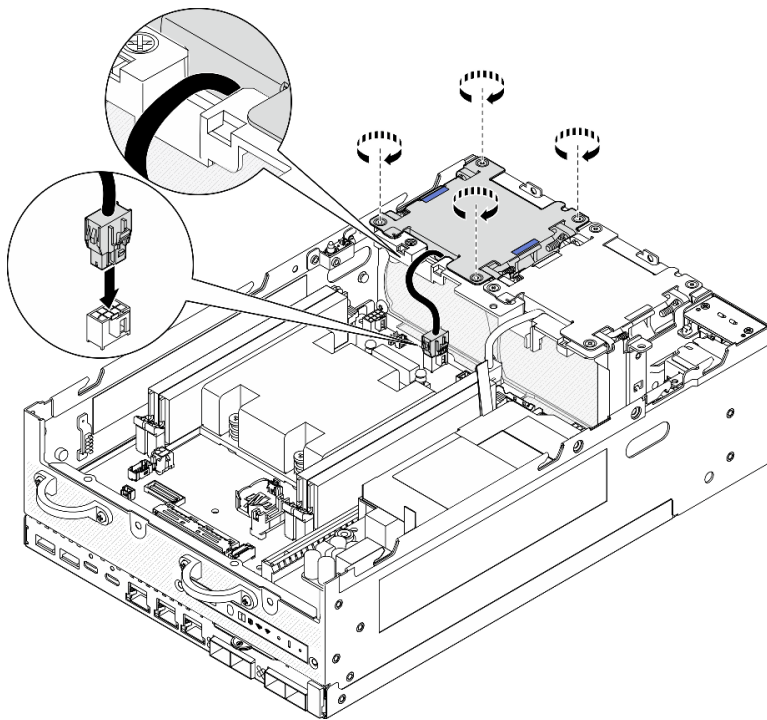
Figura 129. Instalación del módulo de ventilador
