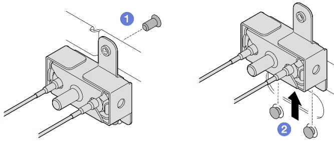
Figura 306. Extracción del conjunto de SMA
