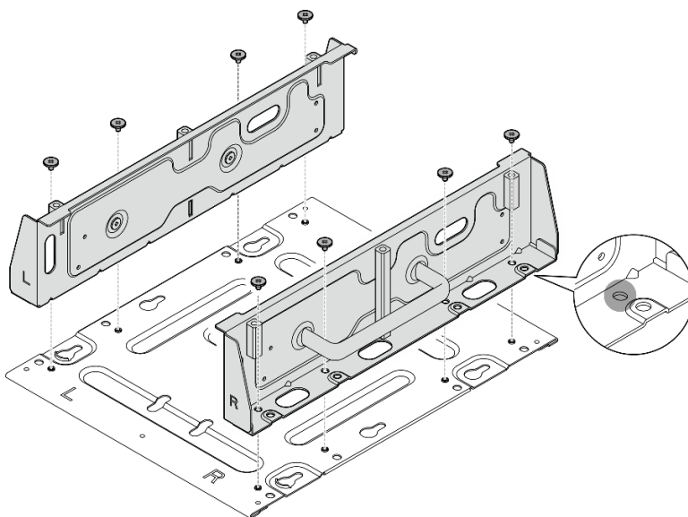
Figura 38. Desensamblaje del soporte del nodo
