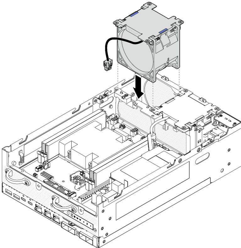
Figura 128. Instalación del módulo de ventilador
