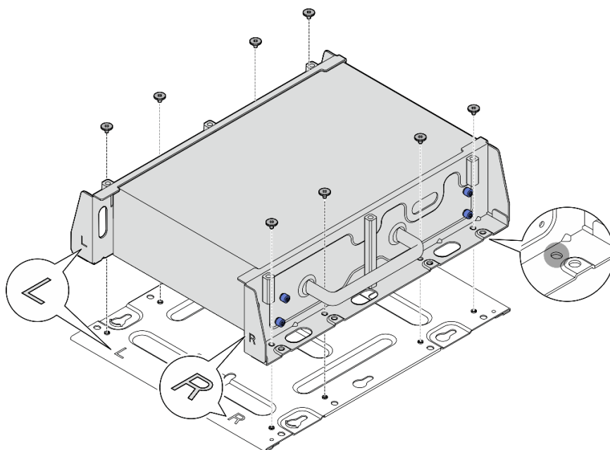
Figura 62. Instalación de la placa inferior
