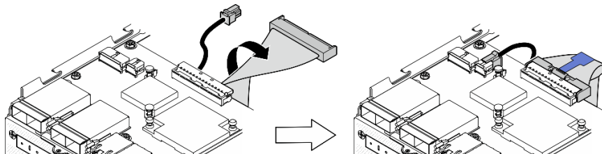
Figura 161. Conexión de los cables de la placa de E/S
