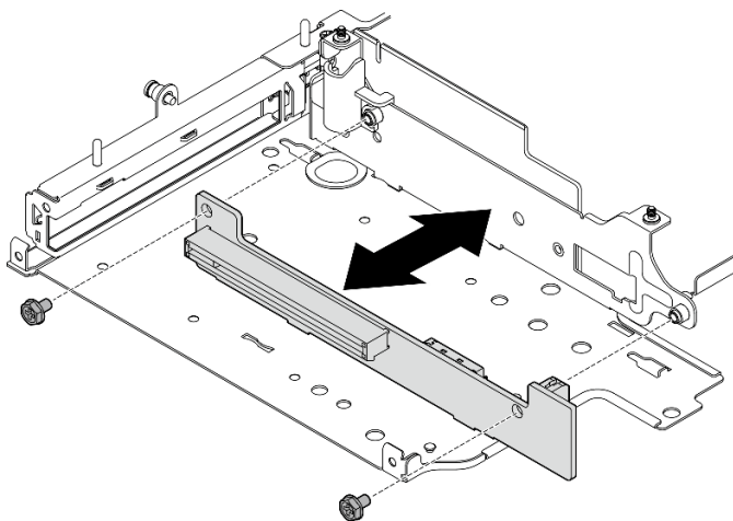
Figura 228. Extracción de la tarjeta de expansión
