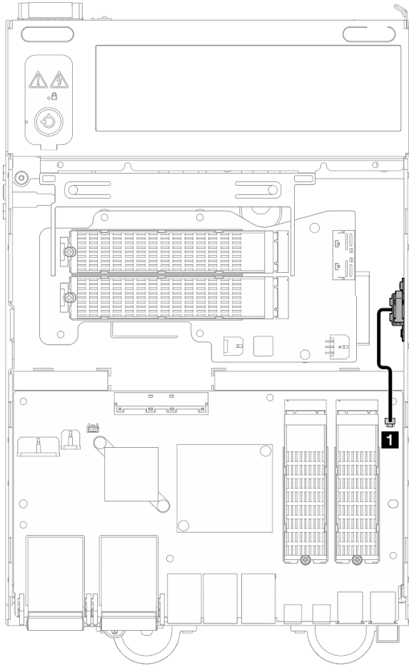
Figura 153. Disposición de los cables del conmutador de intrusión inferior
