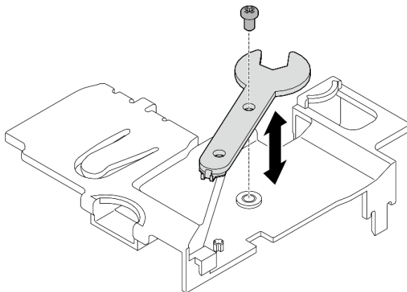
Figura 111. Almacenamiento de la llave
