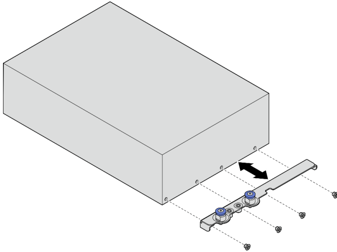
Figura 20. Instalación del soporte del alojamiento
