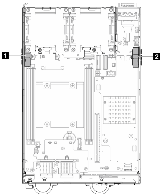
Figura 323. Ubicaciones del conjunto de SMA
