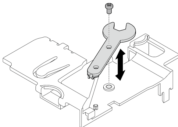
Figura 322. Desenganche de la llave
