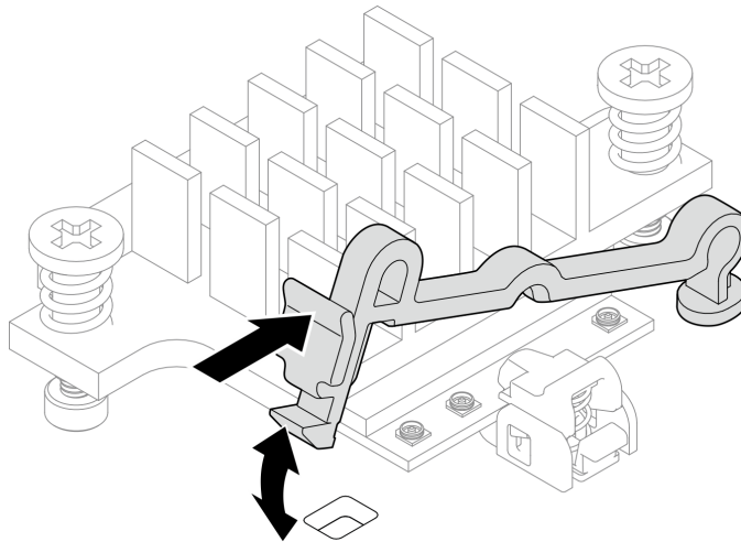
Figura 305. Inserción del soporte de cable
