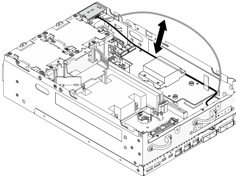
Figura 207. Colocación del cable de señal
