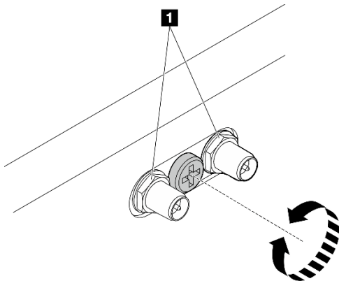
Figura 30. Acortamiento de los conectores SMA
