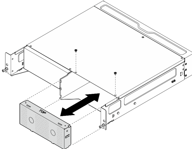
Figura 23. Instalación del relleno del nodo
