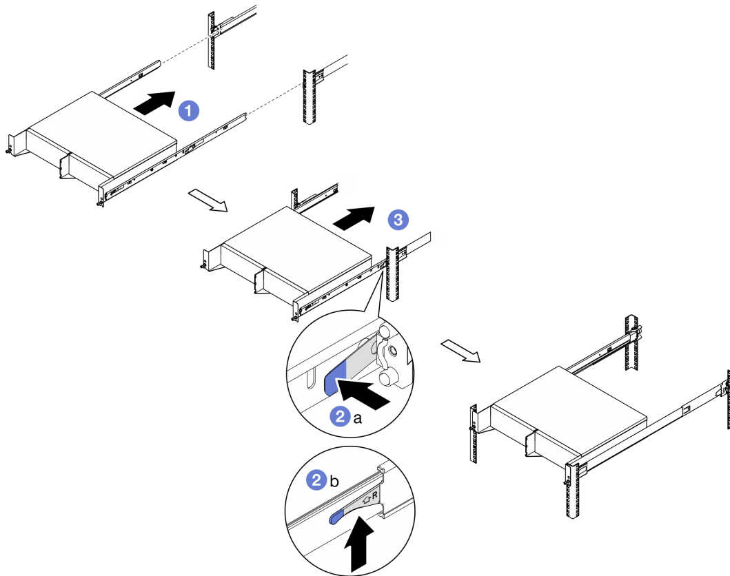
Figura 17. Instalación del alojamiento en el bastidor
