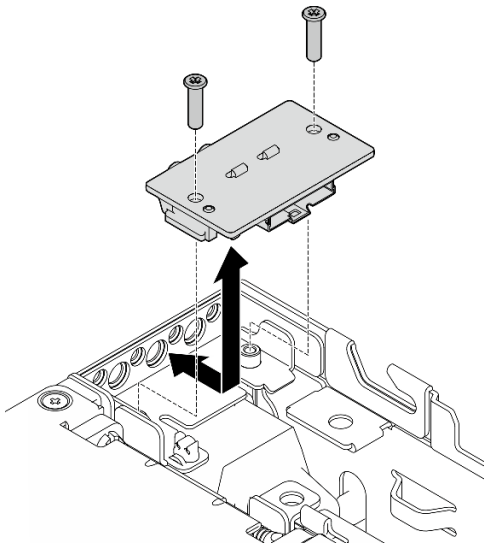
Figura 221. Instalación del panel posterior del operador
