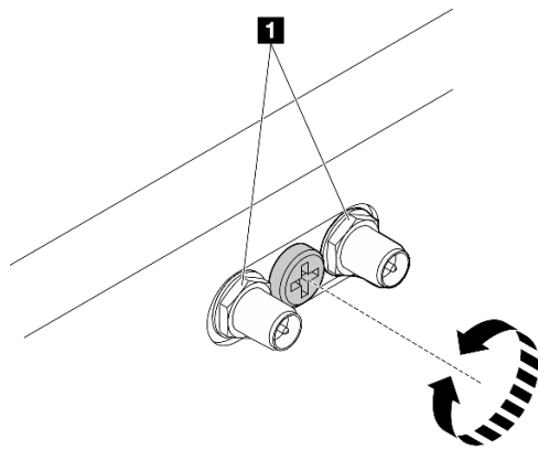
Figura 299. Acortamiento de los conectores SMA
