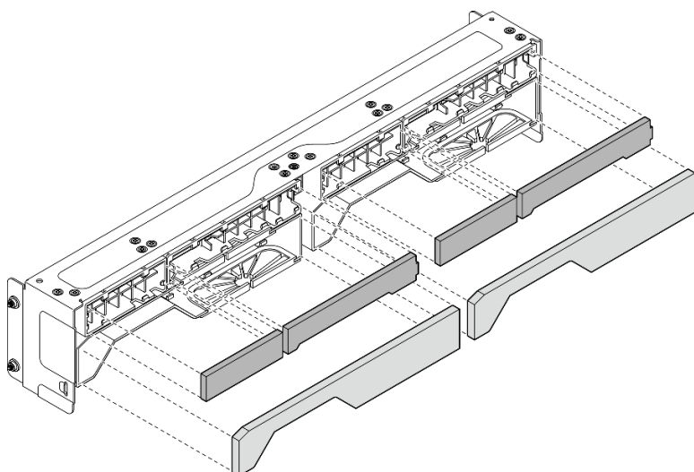
Figura 69. Instalación de los filtros de polvo
