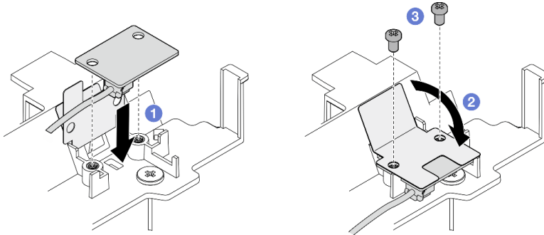
Figura 90. Instalación de la placa del sensor de flujo de aire
