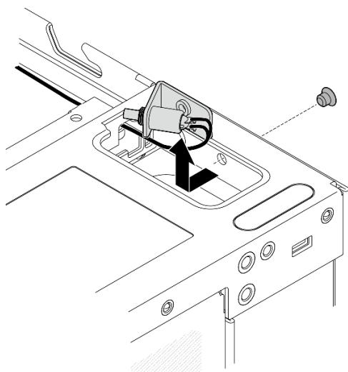
Figura 168. Extracción del conmutador de posición de bloqueo con cable
