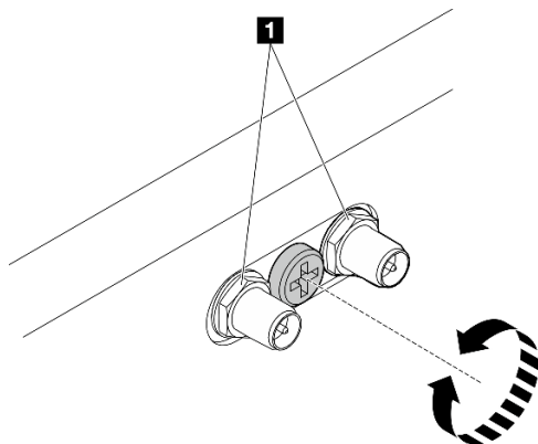
Figura 310. Acortamiento de los conectores SMA
