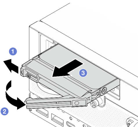
Figura 77. Extracción de una unidad de 7 mm
