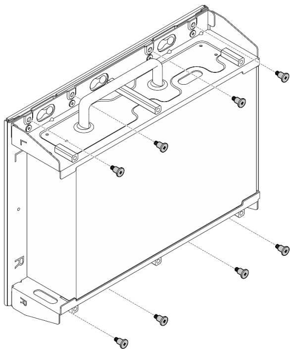
Figura 48. Instalación del soporte del nodo
