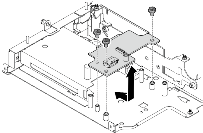
Figura 230. Extracción de la placa posterior 1
