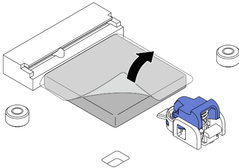
Figura 286. Retirada de la película de la almohadilla térmica
