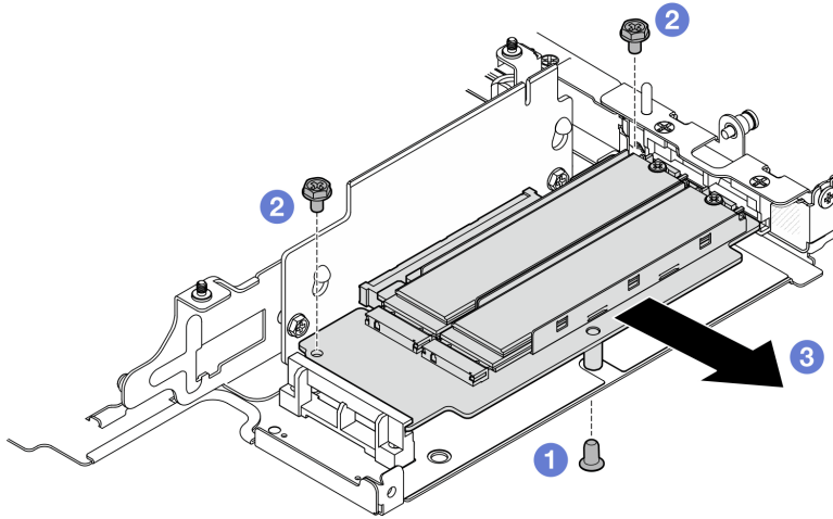
Figura 236. Extracción del adaptador M.2
