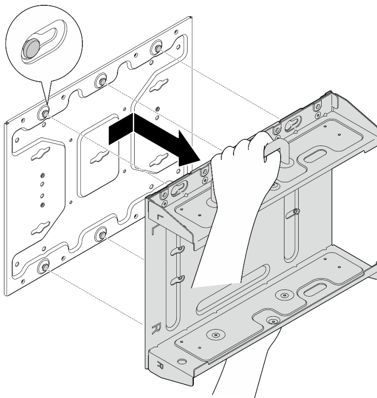
Figura 28. Extracción del soporte del nodo
