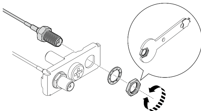
Figura 325. Fijación de los cables al soporte
