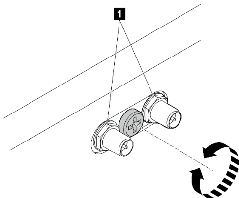
Figura 337. Extensión de los conectores SMA
