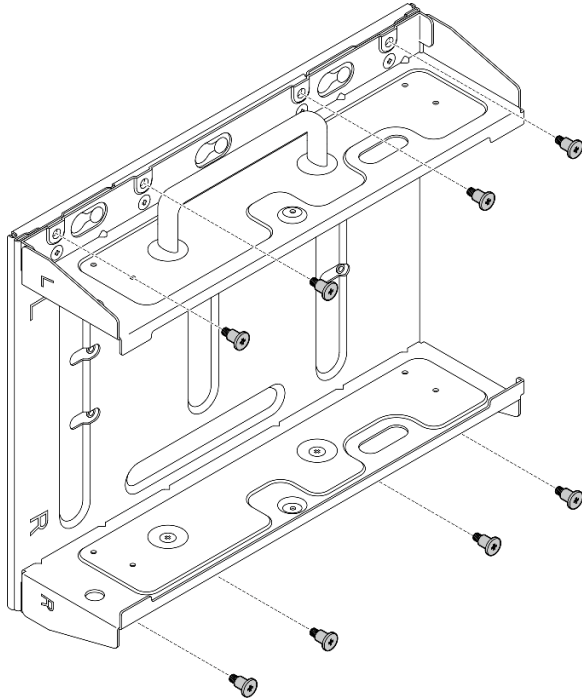
Figura 27. Extracción del soporte del nodo
