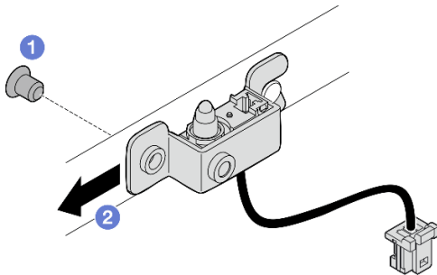
Figura 143. Extracción del conmutador de intrusión con cable
