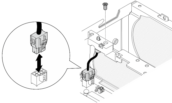
Figura 125. Instalación del conmutador de dirección del ventilador
