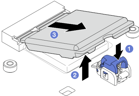
Figura 285. Extracción de la cubierta de relleno
