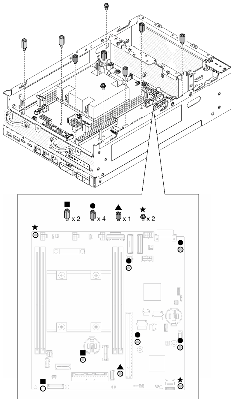
Figura 272. Los tornillos y los separadores de la placa del sistema
