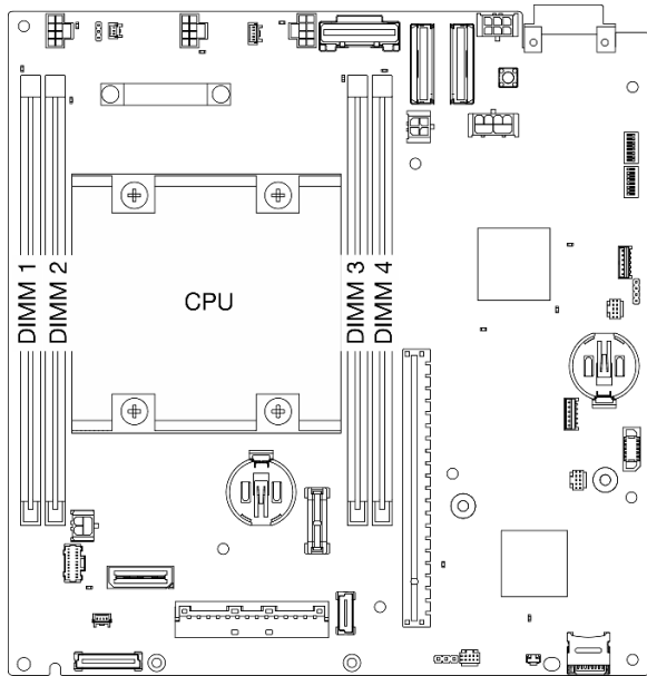
Figura 1. Diseño de los módulos de memoria y el procesador
