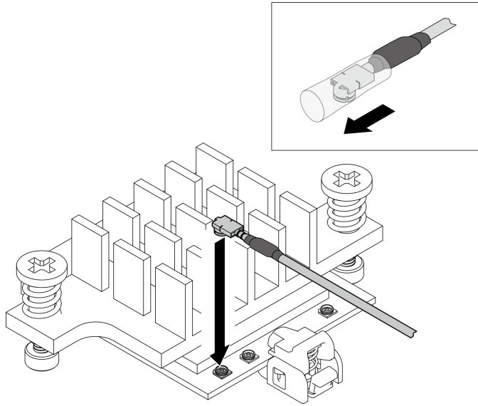
Figura 291. Conexión del cable
