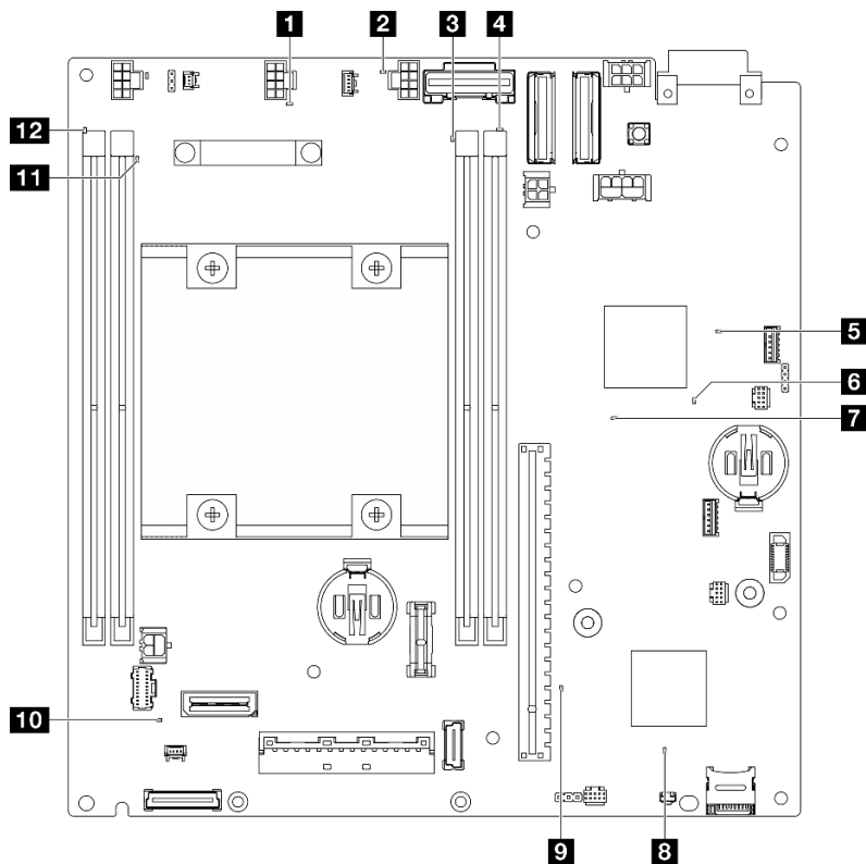
Figura 351. LED de la placa del sistema
