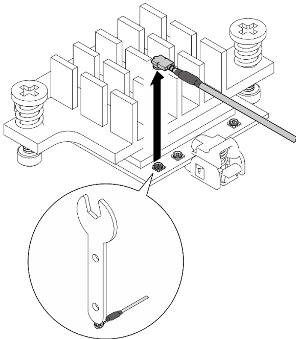
Figura 303. Desconexión del cable
