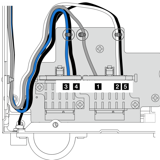
Figura 294. Disposición de los cables para el adaptador inalámbrico
