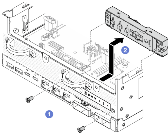
Figura 130. Extracción del panel frontal del operador
