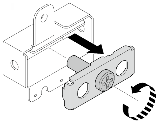
Figura 324. Extracción del soporte
