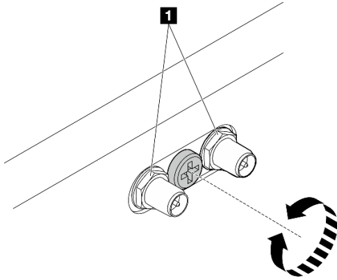
Figura 58. Acortamiento de los conectores SMA
