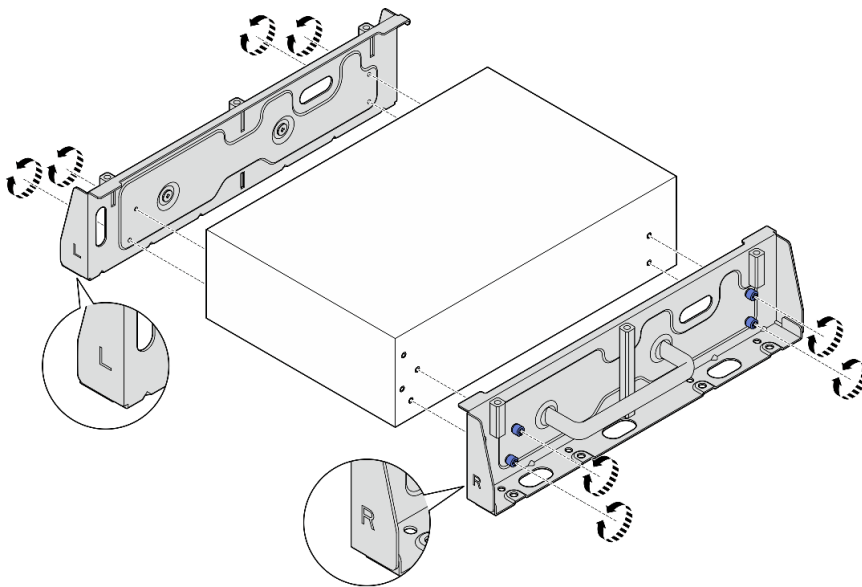
Figura 33. Aflojado de los tornillos ajustables para extraer los soportes laterales
