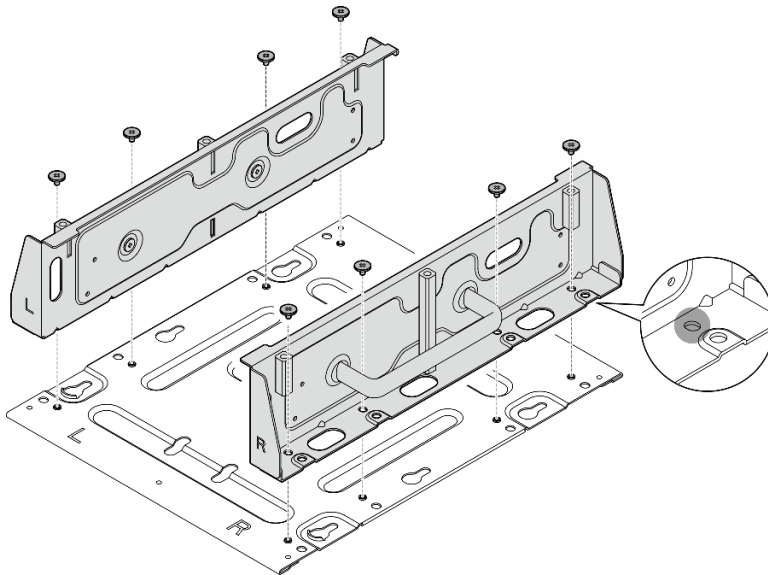
Figura 59. Desensamblaje del soporte del nodo
