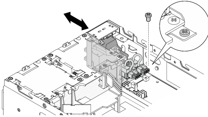
Figura 202. Extracción del módulo PIB de CC
