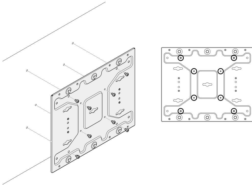
Figura 44. Instalación de la placa de montaje en pared
