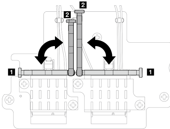
Figura 108. Giro del soporte del cable
