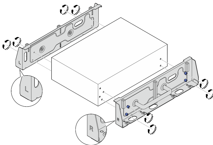
Figura 61. Instalación de los soportes laterales con tornillos ajustables
