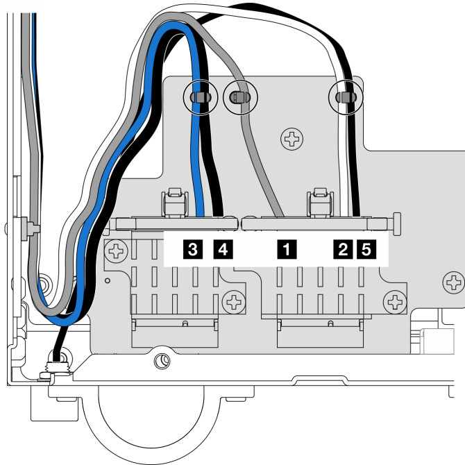
Figura 290. Disposición de los cables para el adaptador inalámbrico
