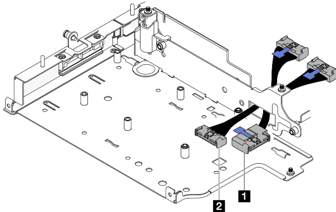
Figura 247. Cable de señal del adaptador con cable M.2
