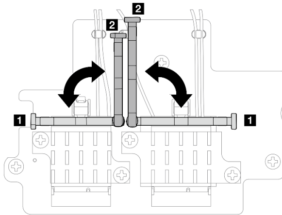
Figura 313. Giro del soporte del cable
