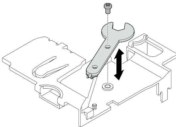
Figura 335. Almacenamiento de la llave
