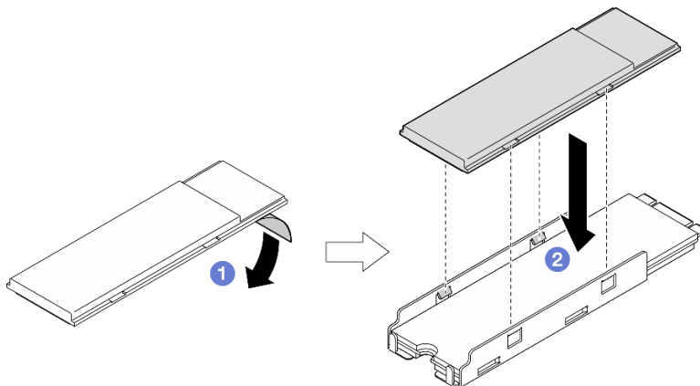
Figura 175. Instalación del disipador de calor M.2
