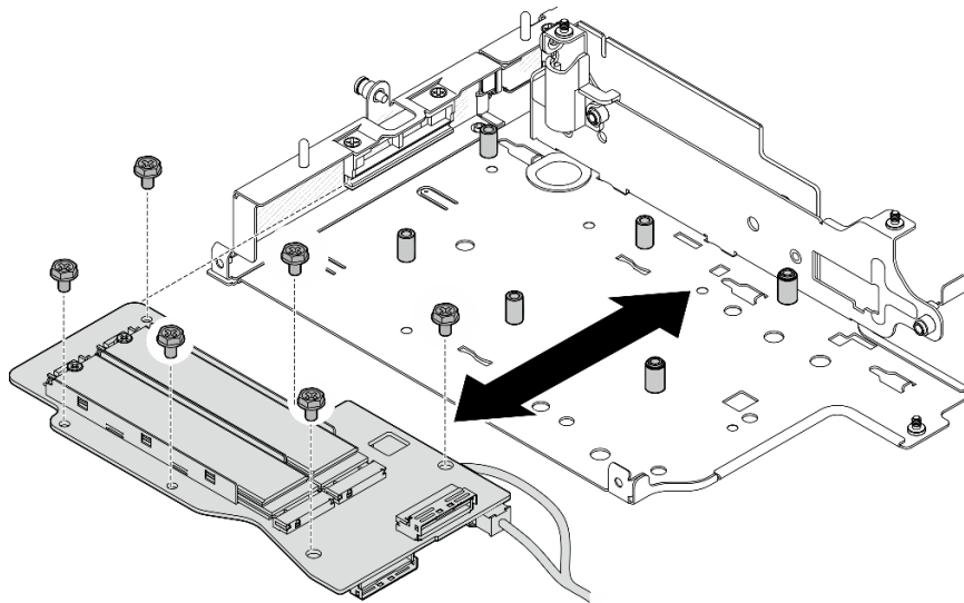
Figura 248. Instalación del adaptador M.2
