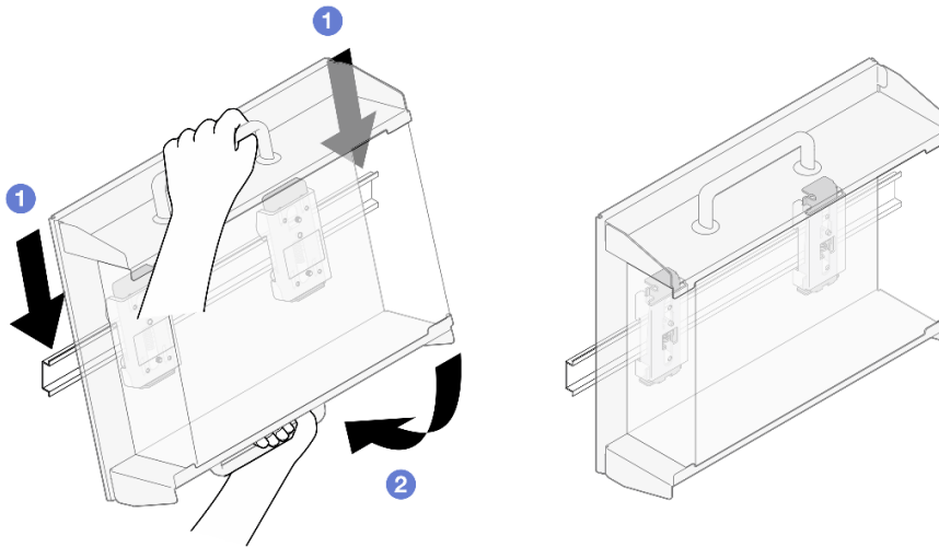
Figura 64. Instalación de la manga del nodo
