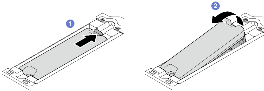
Figura 231. Extracción del módulo de geolocalización
