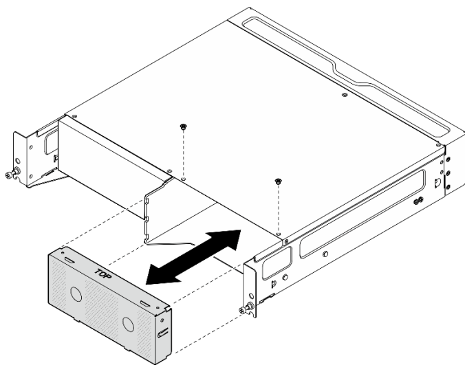
Figura 5. Instalación del relleno del nodo
