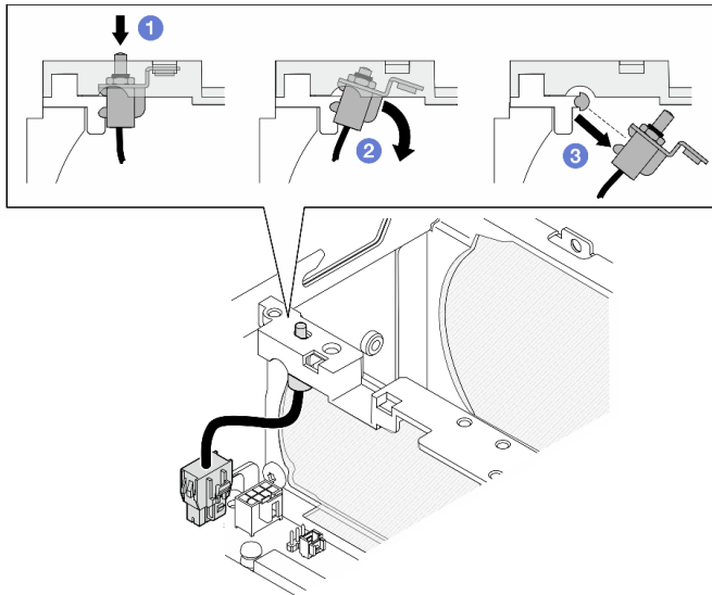
Figura 123. Extracción del conmutador de dirección del ventilador
