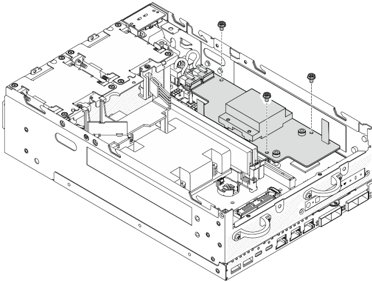
Figura 214. Fijación de la placa del módulo de alimentación
