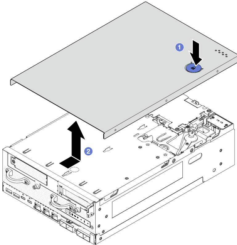
Figura 185. Extracción de la cubierta superior
