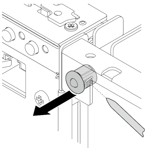
Figura 198. Extracción del cable de LED de estado de PMB
