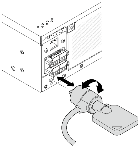
Figura 163. Extracción del candado Kensington
