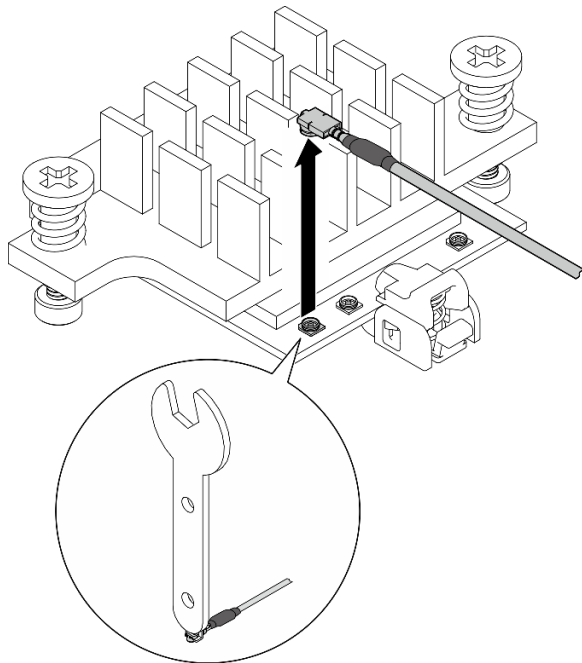
Figura 96. Desconexión del cable
