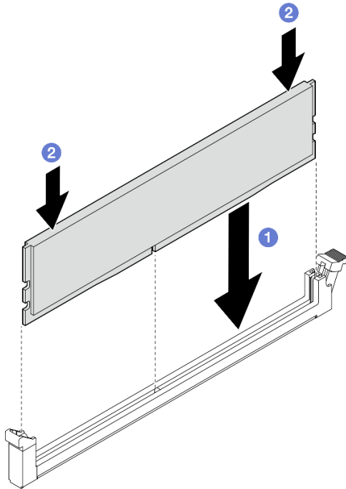
Figura 181. Instalación de un módulo de memoria
