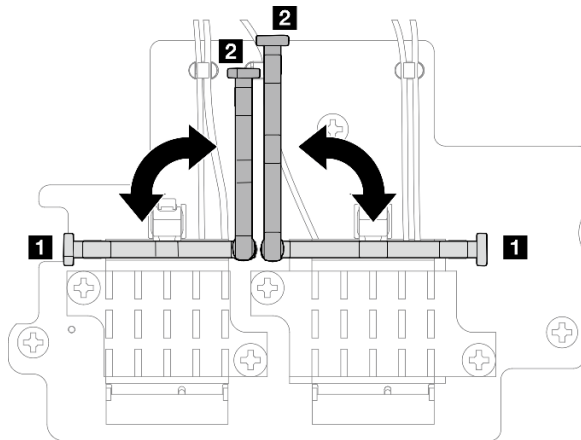
Figura 292. Giro del soporte del cable
