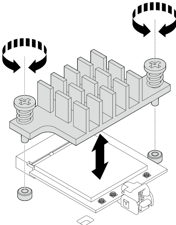
Figura 289. Instalación del disipador de calor del módulo de WLAN/Bluetooth
