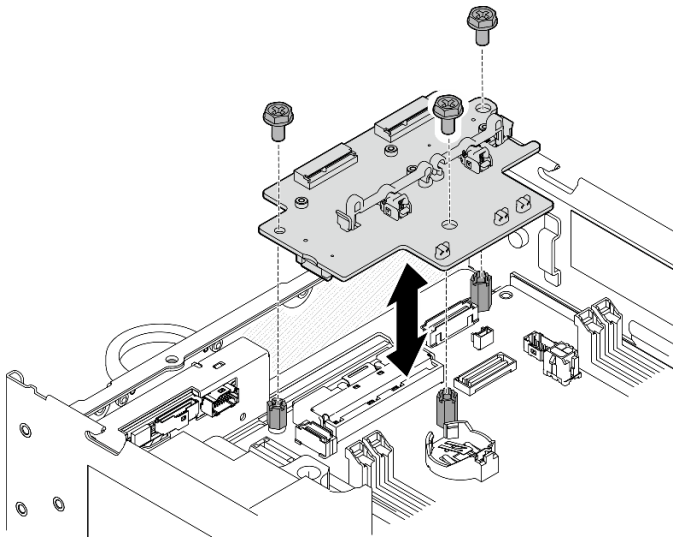
Figura 284. Instalación del adaptador inalámbrico
