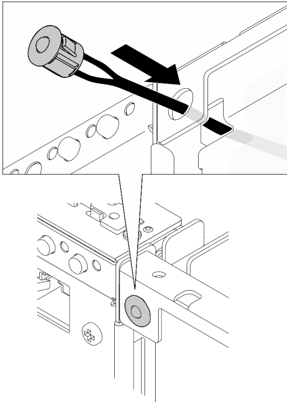
Figura 199. Instalación del cable de LED de estado de PMB
