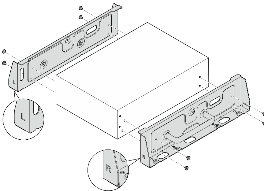
Figura 32. Aflojado de los tornillos para extraer los soportes laterales
