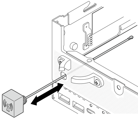
Figura 103. Instalación de la antena Bluetooth
