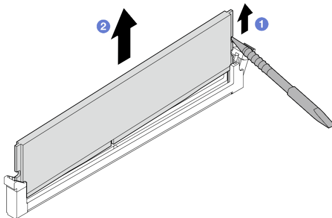
Figura 178. Extracción del módulo de memoria
