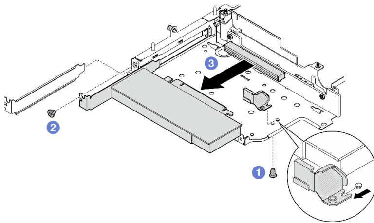
Figura 227. Extracción del adaptador PCIe
