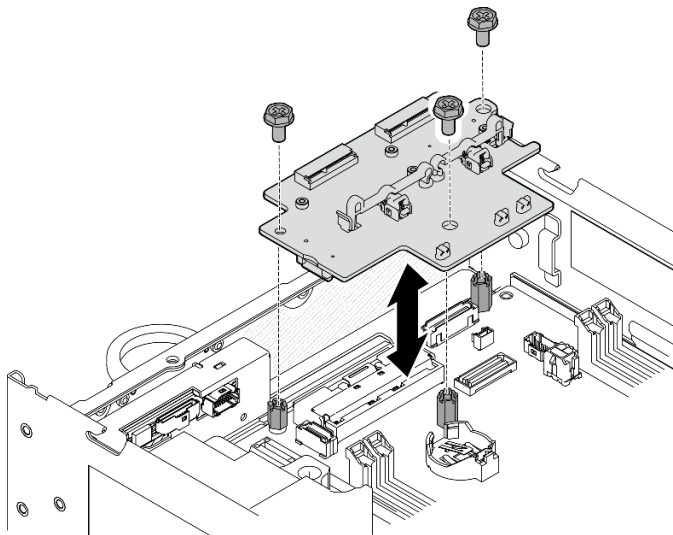
Figura 283. Extracción del adaptador inalámbrico
