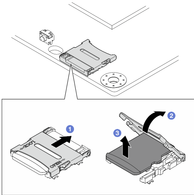
Figura 182. Extraer la tarjeta MicroSD
