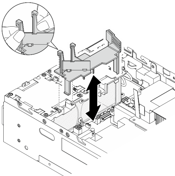
Figura 89. Instalación del deflector de aire
