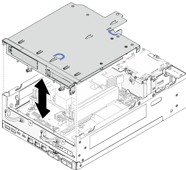
Figura 223. Levantamiento del conjunto de expansión
