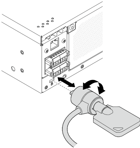
Figura 164. Instalación del candado Kensington
