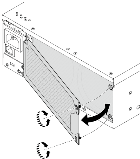
Figura 75. Instalación del marco biselado
