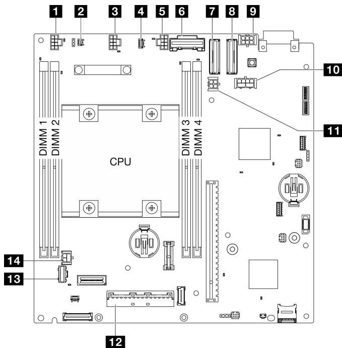
Figura 340. Conectores de la placa del sistema
