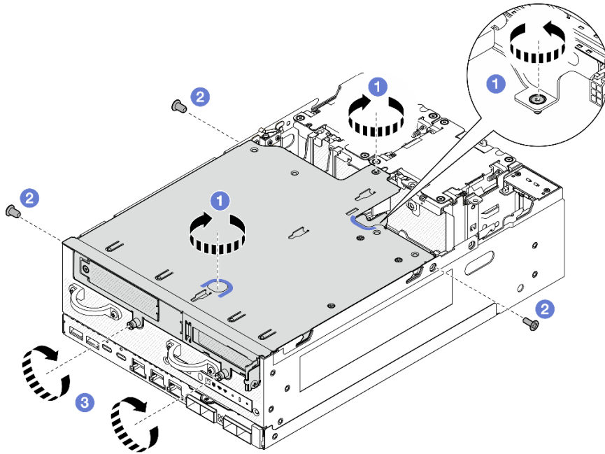
Figura 265. Fijación del conjunto de expansión
