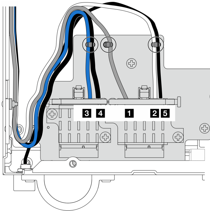
Figura 334. Disposición de los cables para el adaptador inalámbrico
