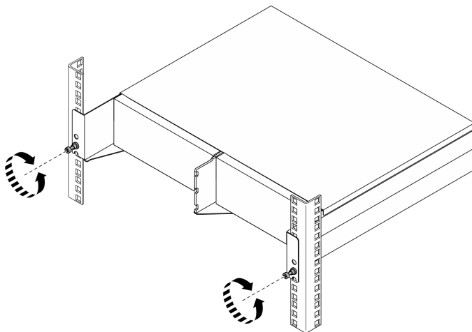
Figura 7. Desenganche del alojamiento del bastidor
