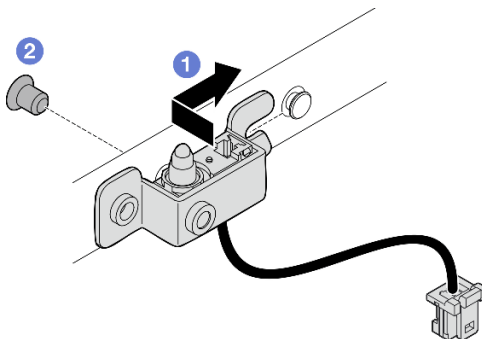
Figura 152. Instalación del conmutador de intrusión con cable
