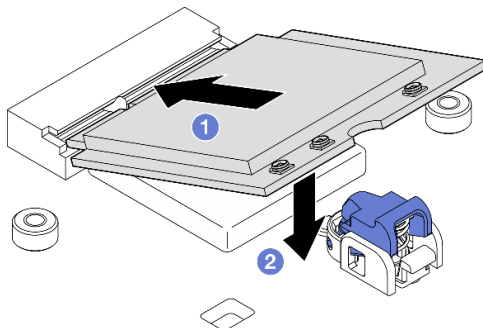
Figura 287. Instalación del módulo de WLAN/Bluetooth
