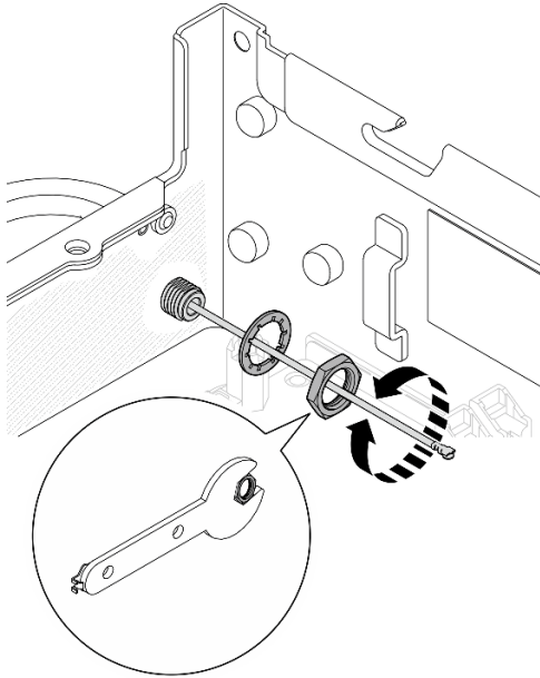
Figura 104. Instalación de la antena Bluetooth
