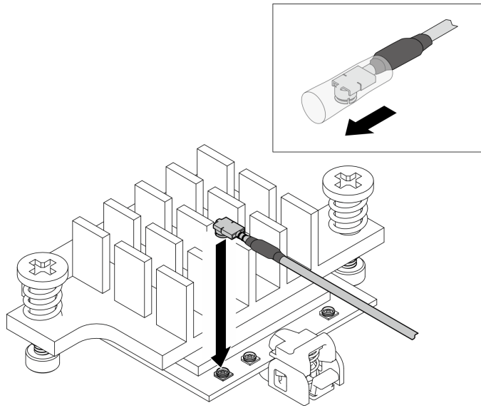
Figura 331. Conexión del cable
