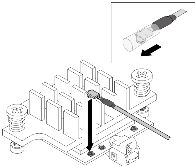
Figura 107. Conexión del cable
