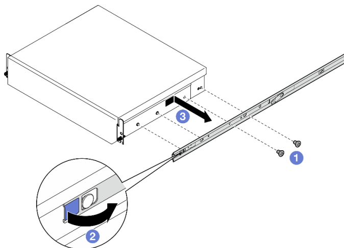
Figura 9. Extracción del riel interno
