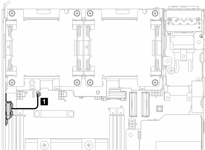
Figura 142. Disposición de los cables del conmutador de intrusión superior
