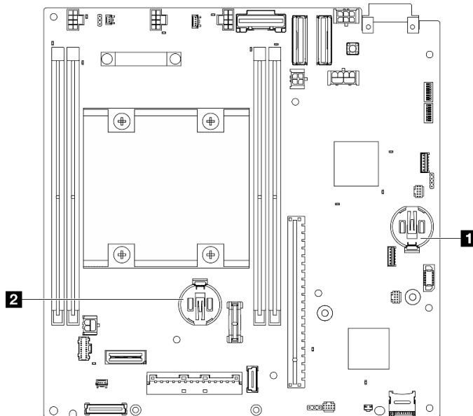
Figura 117. Ubicaciones de la batería de CMOS en la placa del sistema
