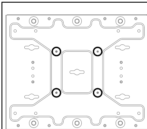
Figura 45. Ubicaciones de los tornillos M4
