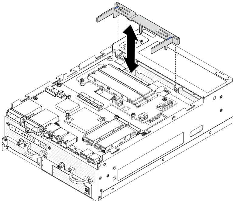
Figura 83. Instalación del deflector de aire
