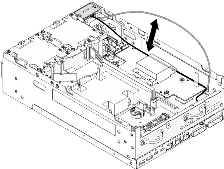
Figura 211. Colocación del cable de señal
