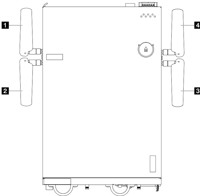
Figura 295. Ubicaciones de las antenas WLAN
