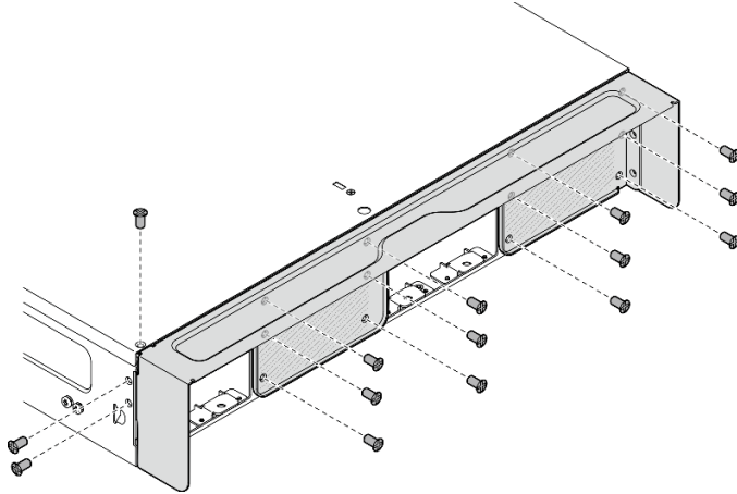
Figura 10. Aflojado de los tornillos
