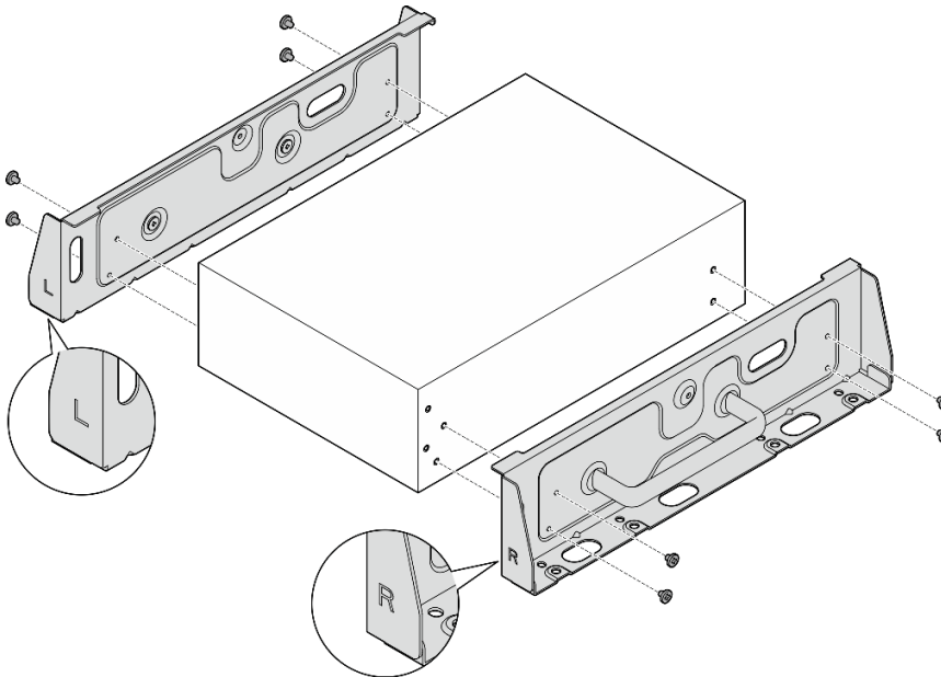
Figura 40. Instalación de los soportes laterales con tornillos
