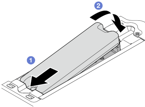
Figura 259. Instalación del módulo de geolocalización
