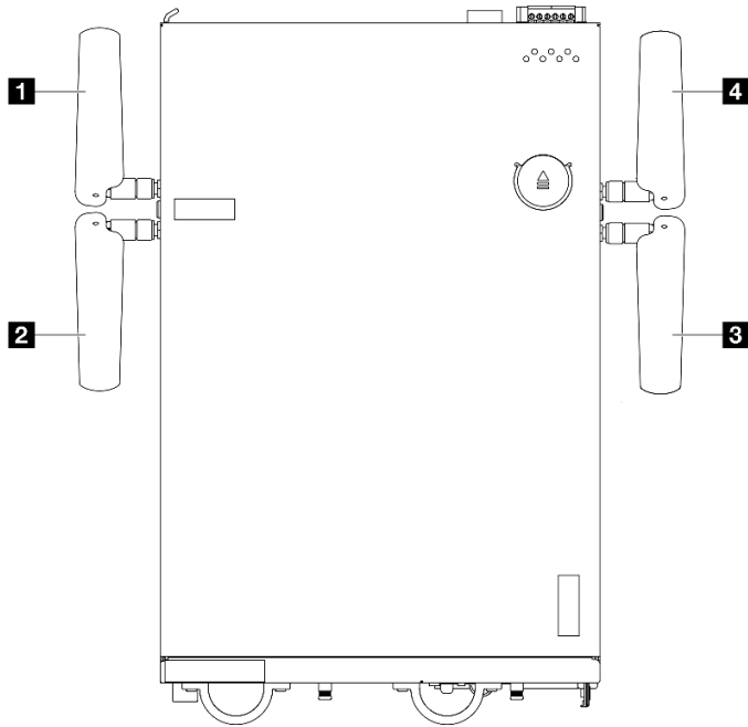
Figura 336. Ubicaciones de las antenas WLAN
