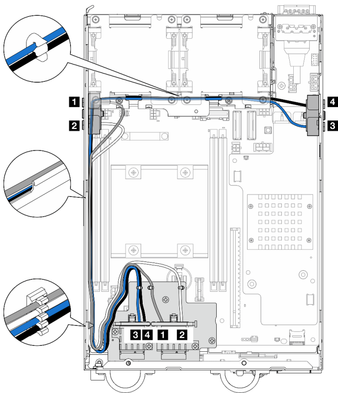
Figura 342. Disposición de los cables de la antena WLAN
