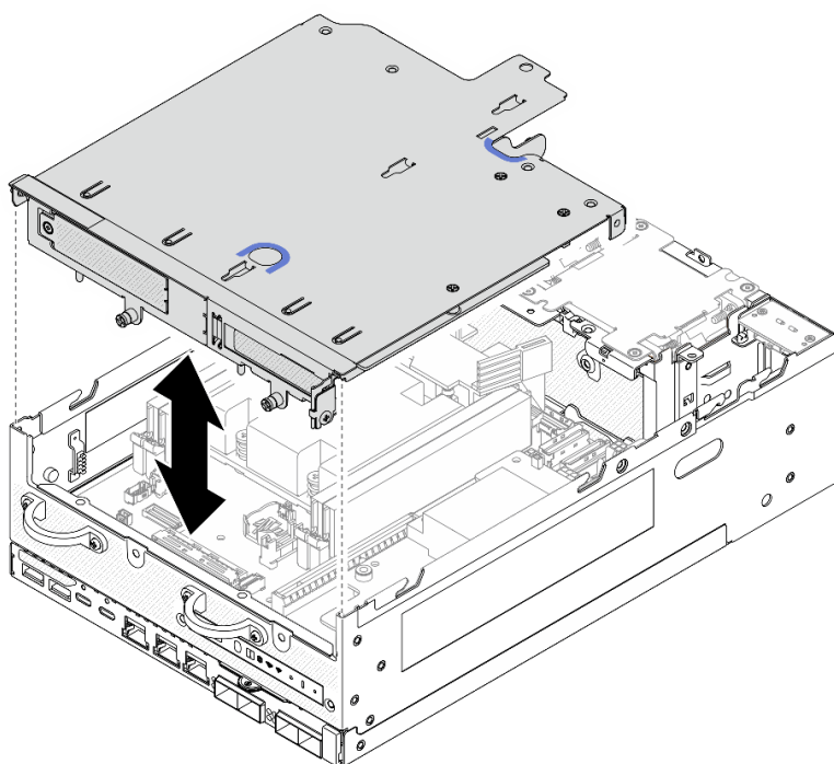
Figura 263. Bajada del conjunto de expansión
