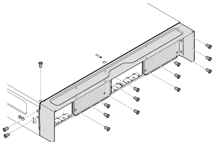
Figura 13. Apriete de los tornillos
