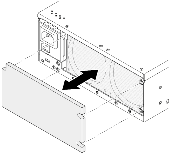
Figura 74. Instalación del filtro de polvo
