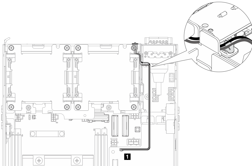
Figura 215. Cable de LED de PMB
