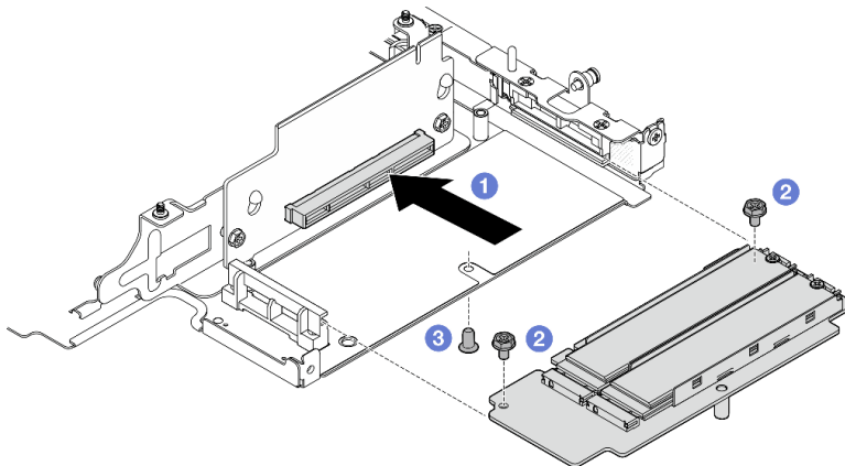
Figura 243. Instalación del adaptador M.2
