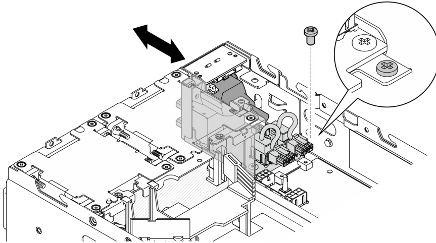
Figura 204. Instalación del módulo PIB
