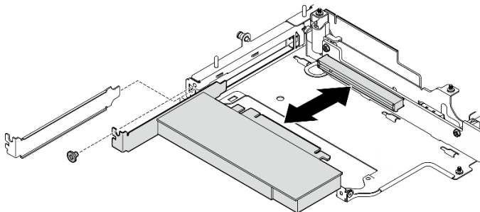
Figura 255. Instalación del adaptador PCIe
