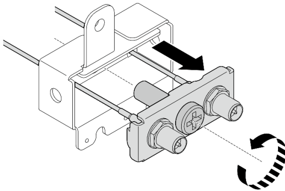
Figura 307. Extracción del soporte
