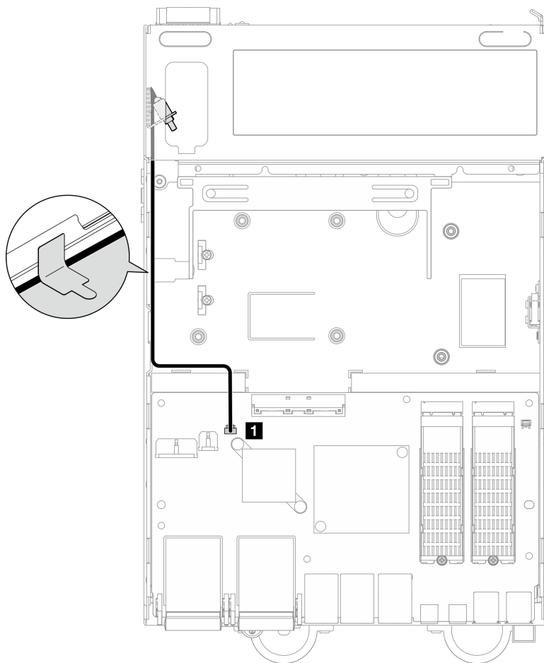
Figura 167. Disposición de los cables del conmutador de posición de bloqueo
