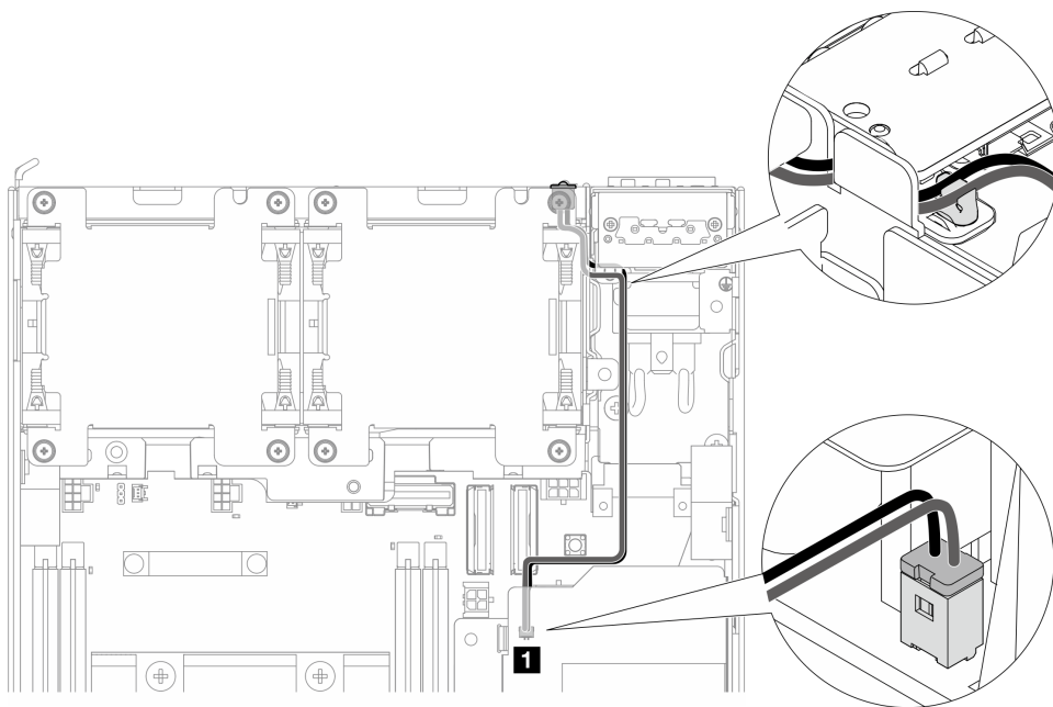
Figura 197. Cable LED de estado de PMB que se conecta a la unidad de fuente de alimentación interna (PMB de CA)
