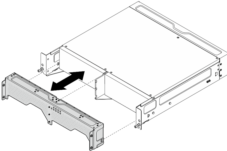
Figura 24. Instalación del soporte de envío
