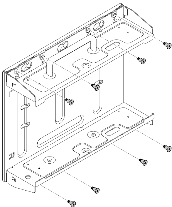
Figura 36. Ensamblaje de la manga del nodo
