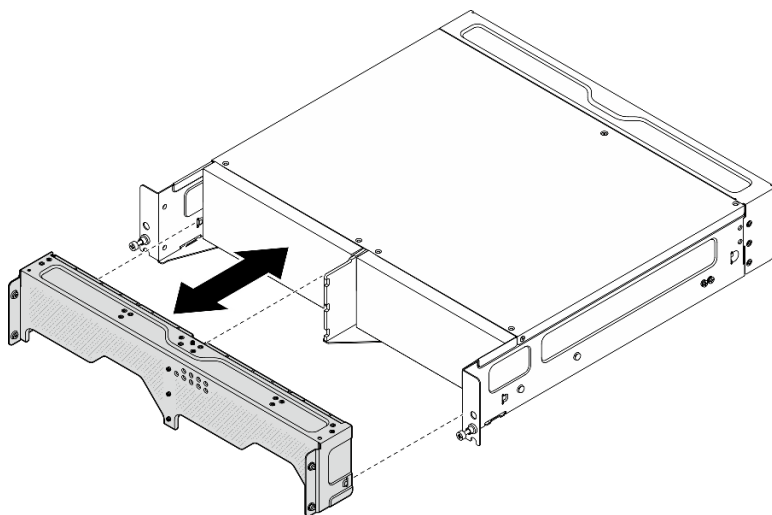
Figura 3. Extracción del soporte de envío
