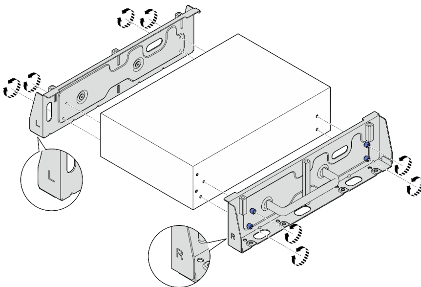
Figura 41. Instalación de los soportes laterales con tornillos ajustables
