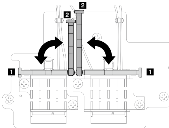
Figura 332. Giro del soporte del cable
