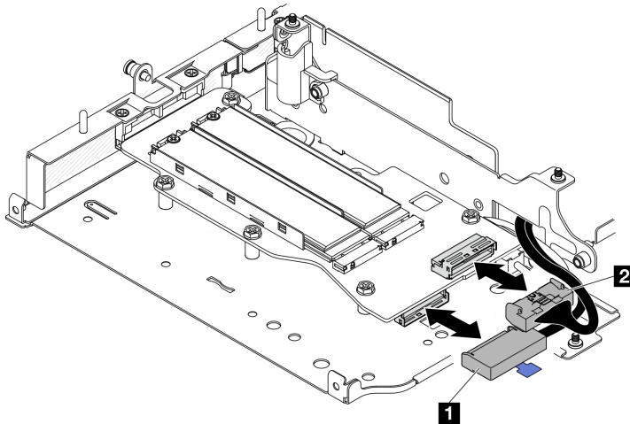
Figura 224. Desconexión del cable de señal
