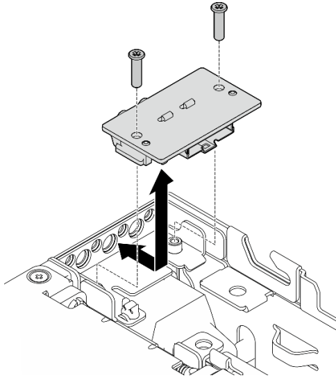
Figura 220. Extracción del panel posterior del operador
