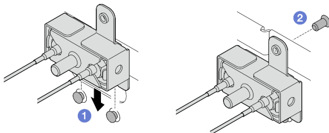
Figura 326. Instalación del conjunto de SMA
