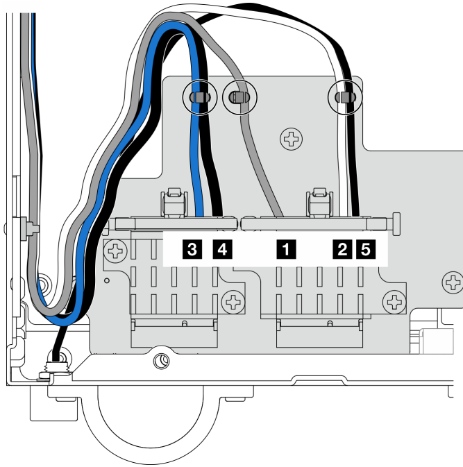
Figura 330. Disposición de los cables para el adaptador inalámbrico
