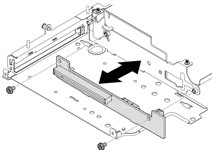
Figura 250. Instalación de la tarjeta de expansión
