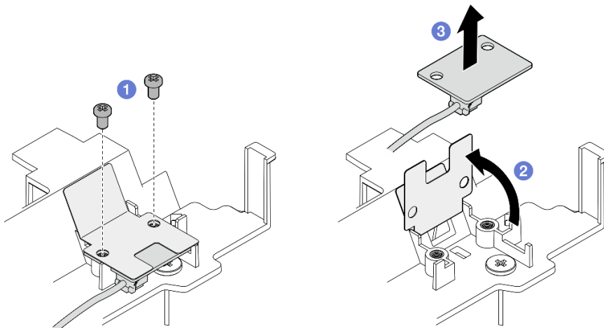
Figura 88. Extracción de la placa del sensor de flujo de aire
