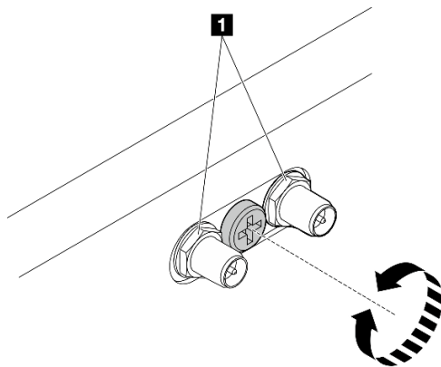
Figura 19. Acortamiento de los conectores SMA
