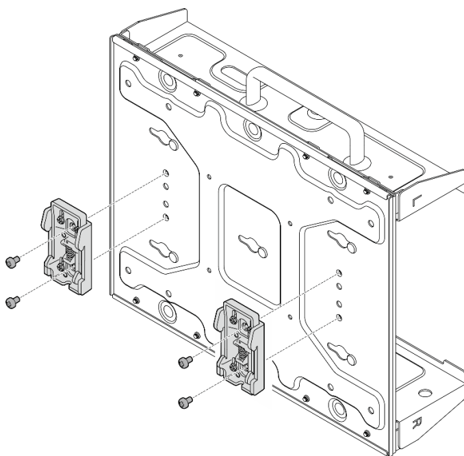
Figura 63. Instalación de los clips del riel DIN
