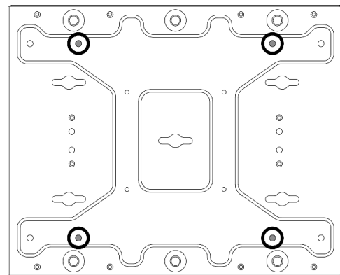
Figura 46. Ubicaciones de los tornillos M6
