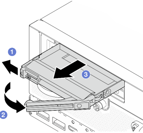
Figura 78. Extracción de un relleno de unidad
