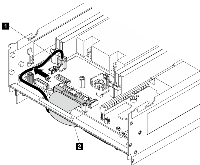
Figura 157. Disposición de los cables de la placa de E/S
