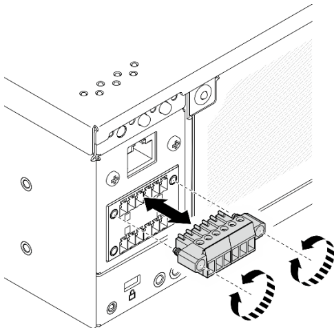
Figura 205. Extracción del cabezal
