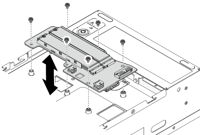
Figura 115. Instalación del adaptador con cable M.2 inferior
