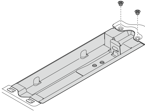
Figura 258. Instalación del compartimiento del módulo de geolocalización
