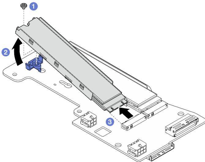
Figura 112. Extracción de una unidad M.2
