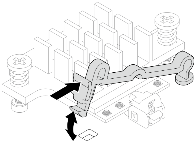
Figura 94. Levantamiento del soporte del cable
