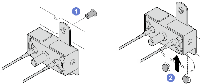
Figura 317. Extracción del conjunto de SMA
