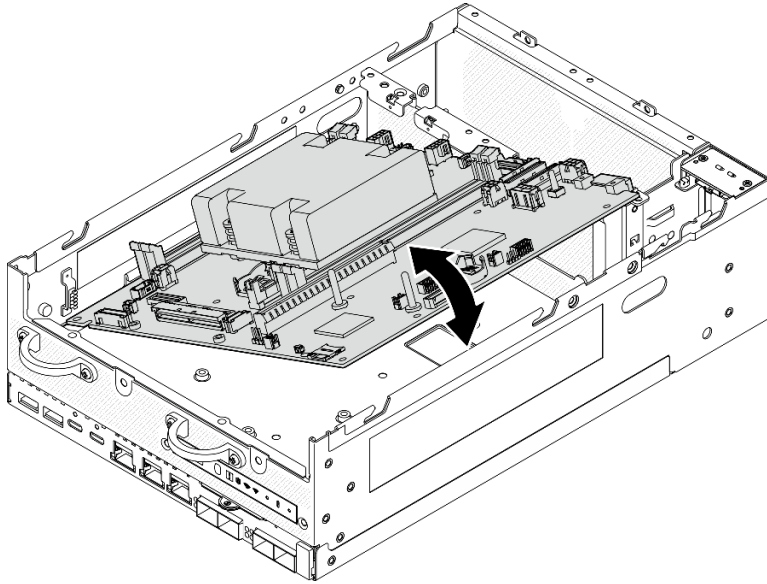
Figura 273. Extracción la placa del sistema
