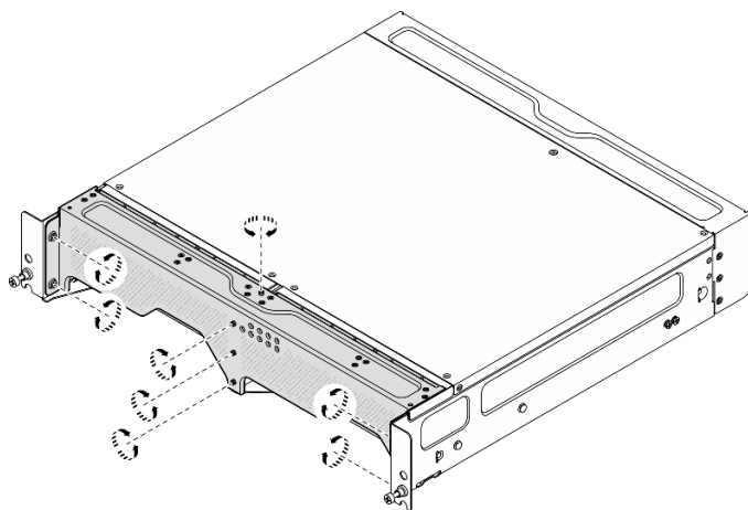
Figura 71. Apriete de los tornillos
