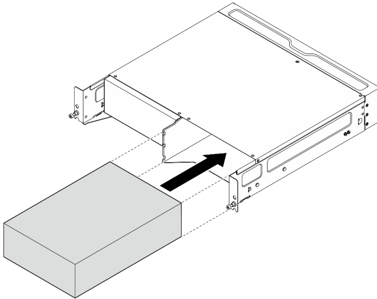
Figura 22. Instalación del nodo
