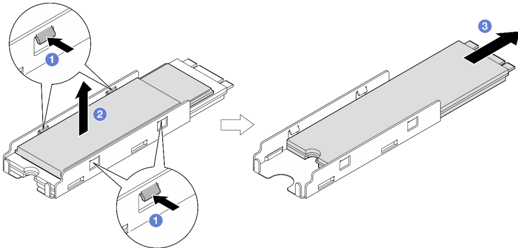
Figura 173. Extracción del disipador de calor M.2
