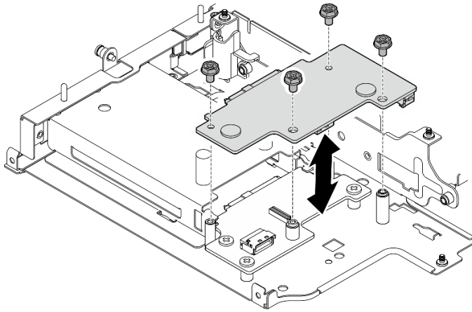
Figura 253. Instalación de la placa posterior 2
