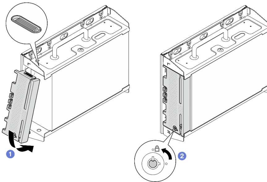
Figura 49. Instalación del marco biselado de seguridad
