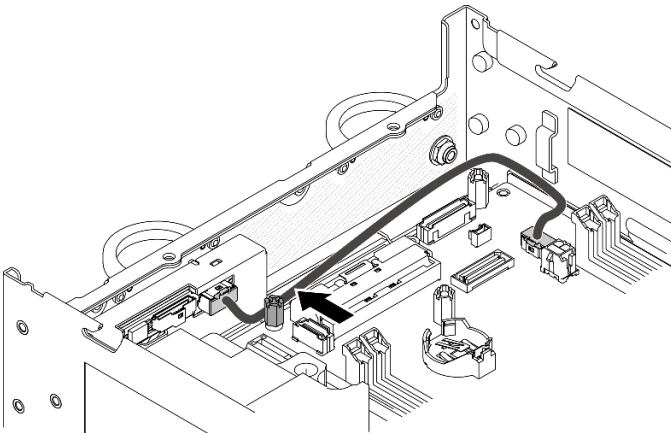
Figura 341. Disposición de los cables del panel frontal del operador
