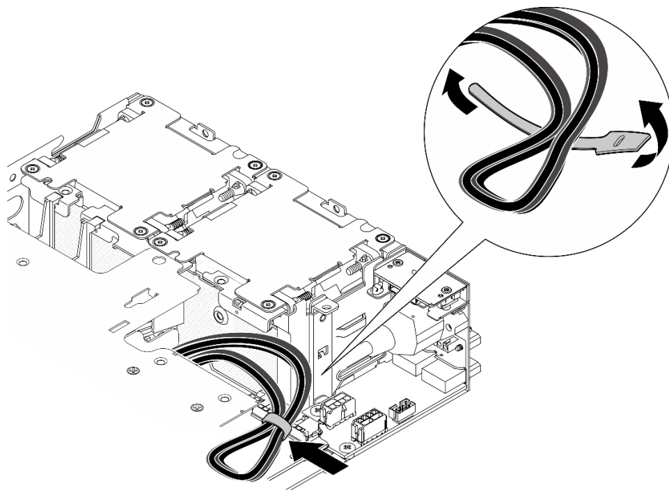
Figura 262. Disposición de los cables para el conjunto de expansión
