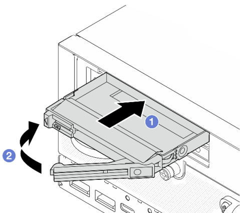
Figura 80. Instalación de un relleno de unidad
