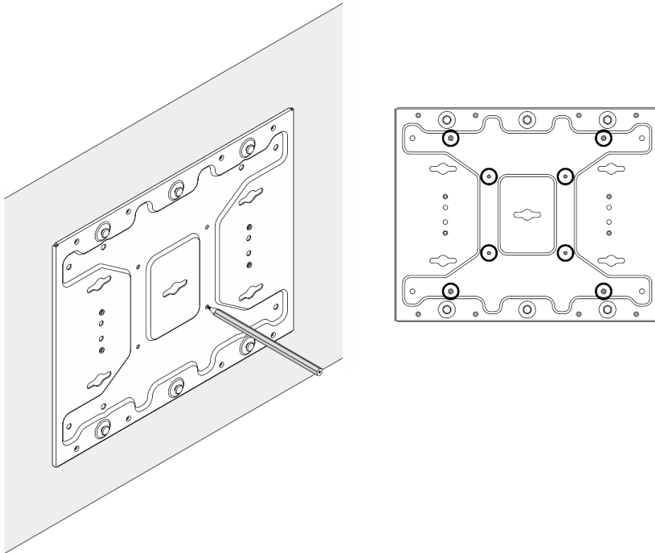
Figura 43. Ubicaciones de los orificios de tornillos
