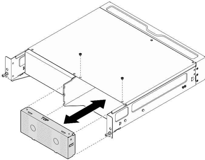
Figura 21. Extracción del relleno del nodo
