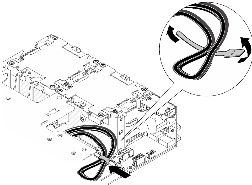
Figura 269. Disposición de los cables para el conjunto de expansión
