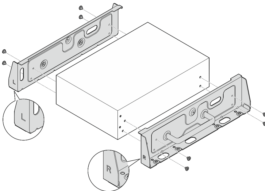
Figura 60. Instalación de los soportes laterales con tornillos
