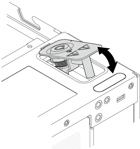
Figura 166. Extracción del bloqueo de seguridad del sistema
