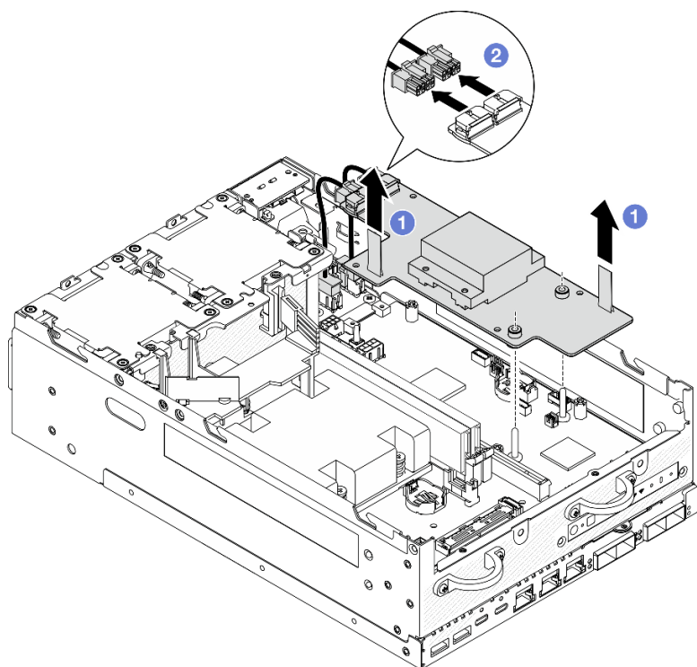
Figura 210. Extracción de la placa del módulo de alimentación
