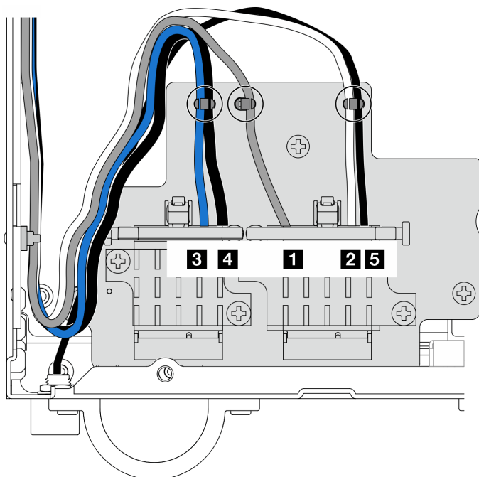
Figura 343. Disposición de los cables de la antena WLAN y Bluetooth
