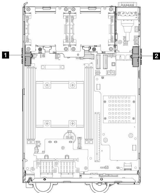
Figura 297. Ubicaciones del conjunto de SMA
