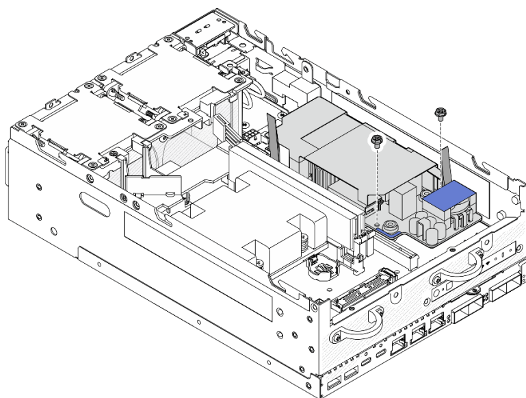
Figura 139. Apriete de los tornillos
