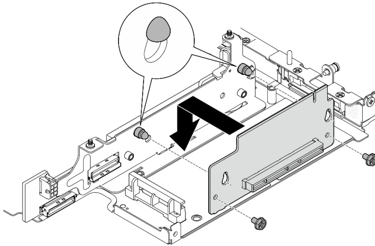
Figura 242. Instalación de la tarjeta de expansión
