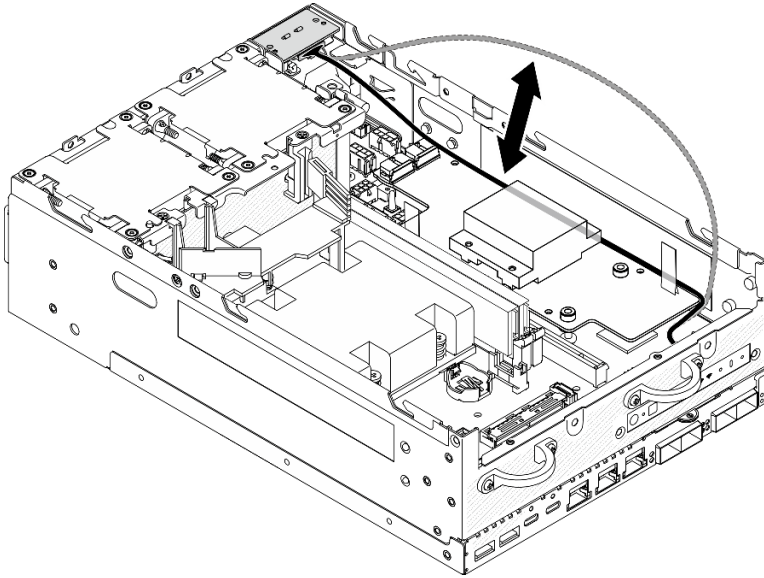
Figura 216. Colocación del cable de señal
