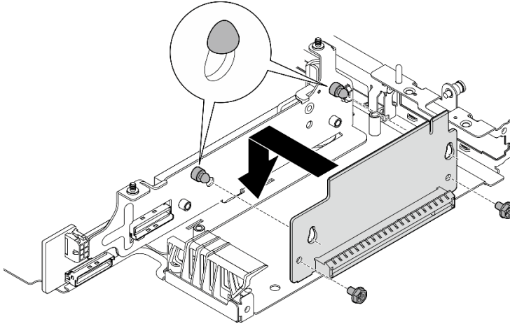
Figura 244. Instalación de la tarjeta de expansión
