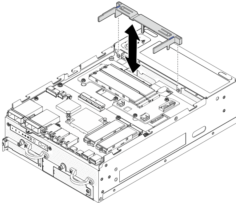
Figura 82. Extracción del deflector de aire
