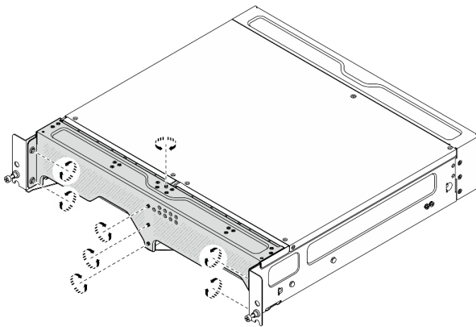
Figura 25. Apriete de los tornillos
