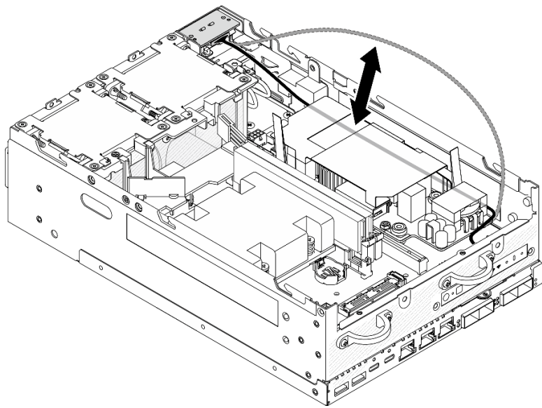
Figura 132. Colocación del cable de señal
