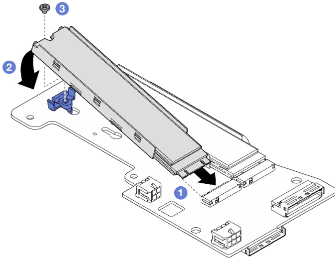
Figura 116. Instalación de una unidad M.2
