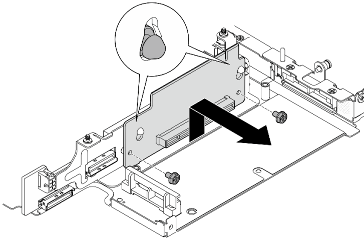
Figura 237. Extracción de la tarjeta de expansión
