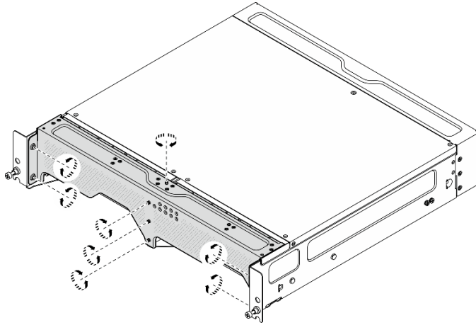
Figura 66. Aflojado de los tornillos
