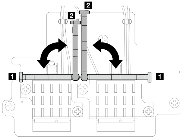
Figura 302. Giro del soporte del cable
