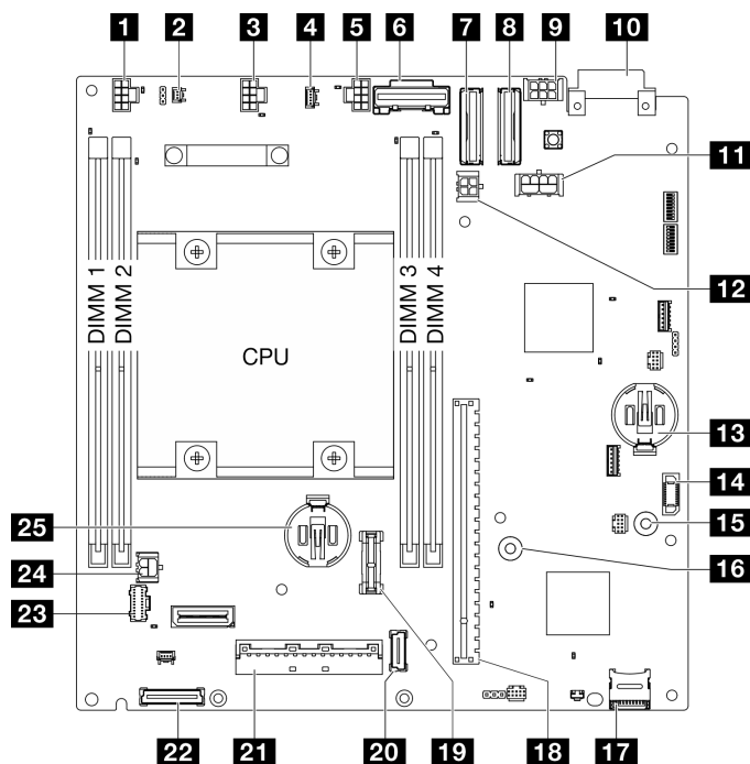
Figura 346. Conectores de la placa del sistema
