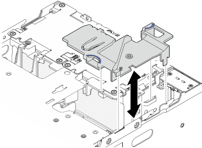
Figura 84. Extracción del deflector de aire
