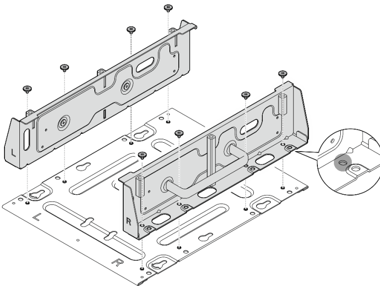
Figura 34. Ensamblaje de la manga del nodo
