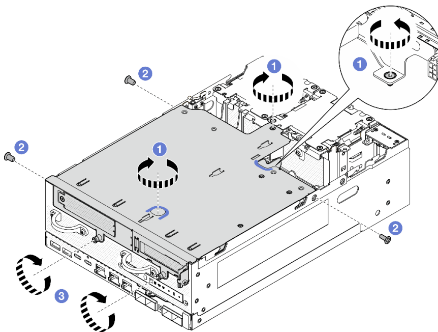
Figura 261. Fijación del conjunto de expansión
