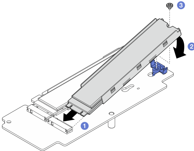
Figura 241. Instalación de una unidad M.2
