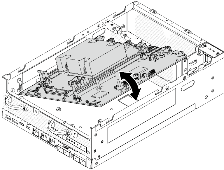
Figura 274. Instalación de la placa del sistema
