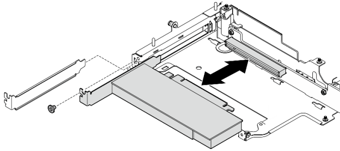
Figura 234. Extracción del adaptador PCIe
