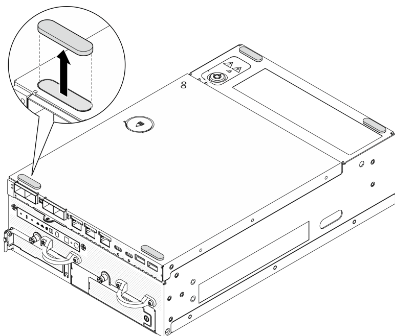
Figura 270. Extracción de las patas de goma
