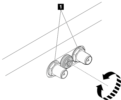
Figure 52. Raccourcissement des connecteurs SMA
