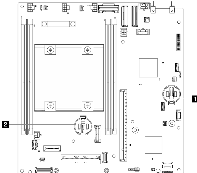
Figure 117. Emplacements de la pile CMOS sur la carte mère
