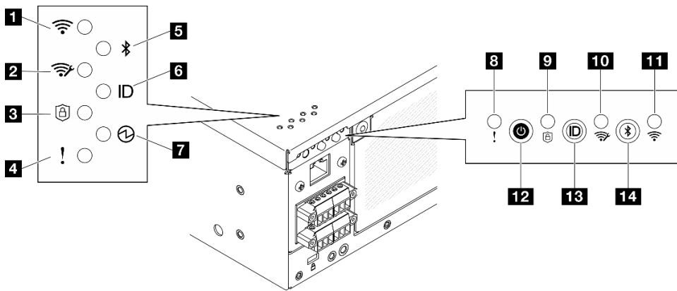
Figure 350. Voyants du panneau opérateur arrière
