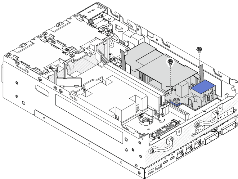
Figure 135. Desserer les vis
