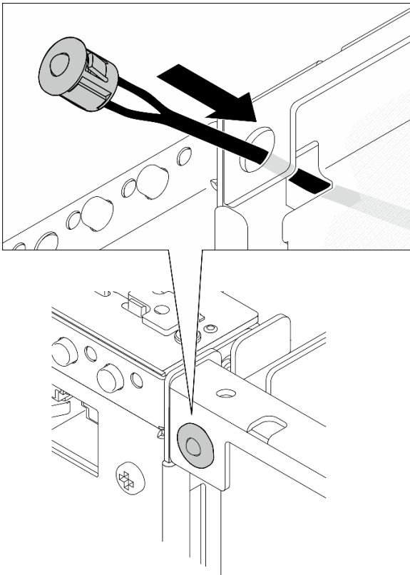
Figure 199. Installation du câble du voyant d'état PMB
