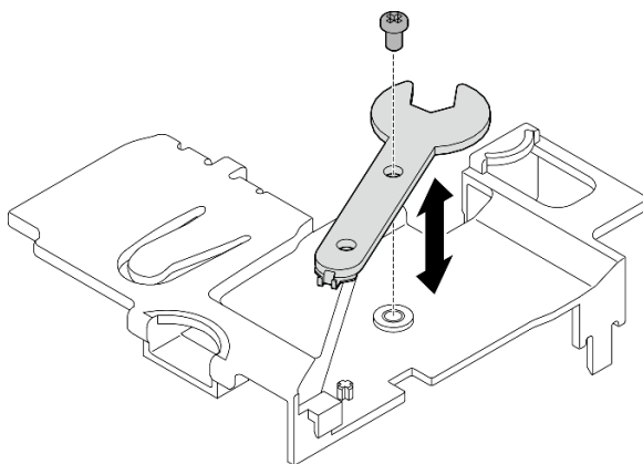
Figure 111. Rangement de la clé
