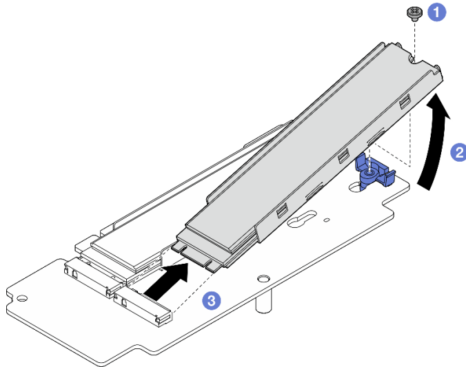
Figure 238. Retrait d'une unité M.2
