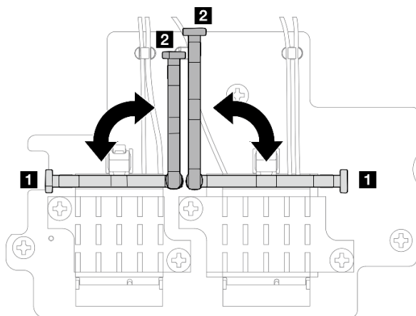
Figure 315. Faire pivoter le support de câble
