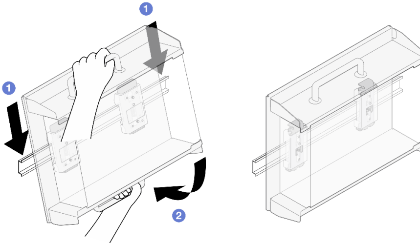
Figure 64. Installation d'un manchon de nœud
