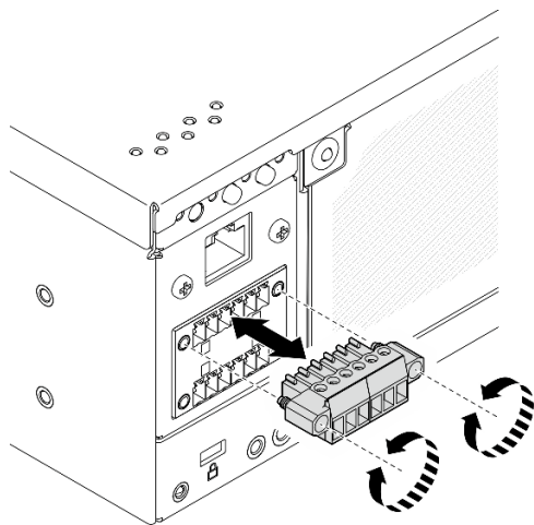
Figure 205. Retrait de l'embase
