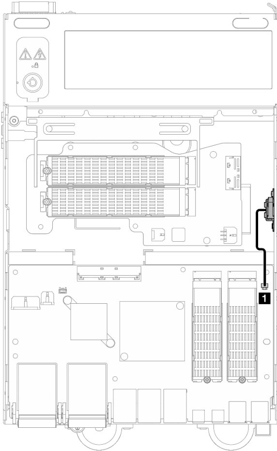
Figure 153. Cheminement des câbles du commutateur d'intrusion inférieur
