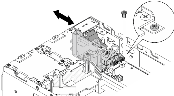
Figure 202. Retrait du module PIB CC
