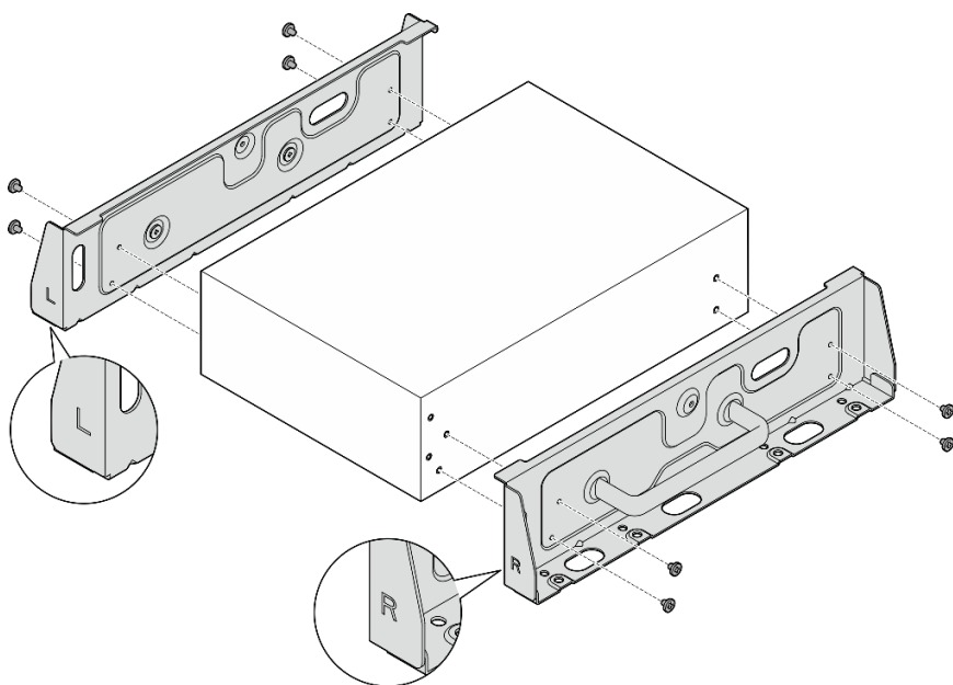
Figure 55. Desserrage des vis pour retirer les supports latéraux
