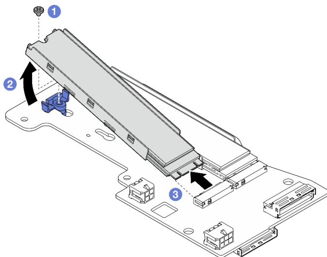
Figure 112. Retrait d'une unité M.2
