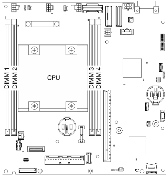
Figure 179. Disposition des modules de mémoire et des processeurs
