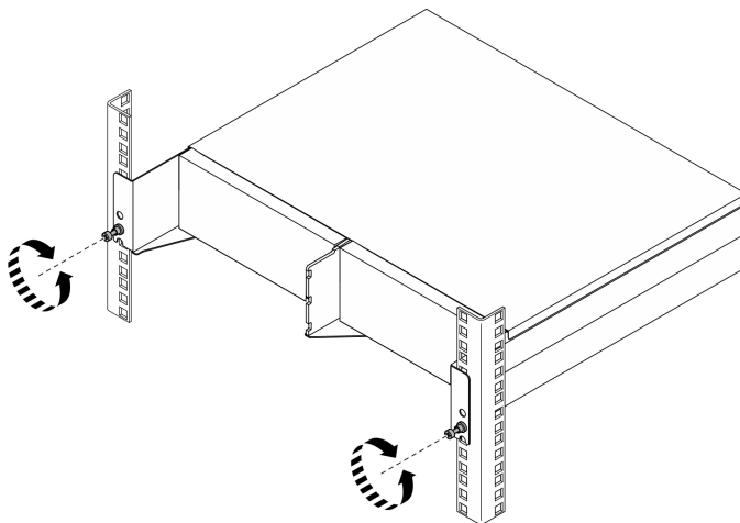
Figure 7. Dégagement du boîtier de l'armoire
