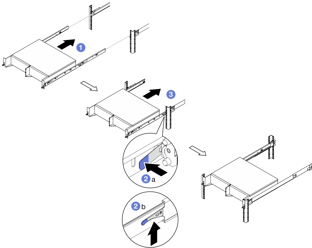
Figure 17. Installation du boîtier dans l'armoire
