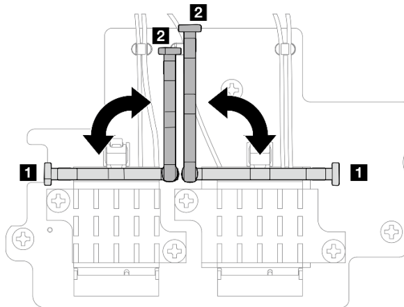
Figure 279. Faire pivoter le support de câble
