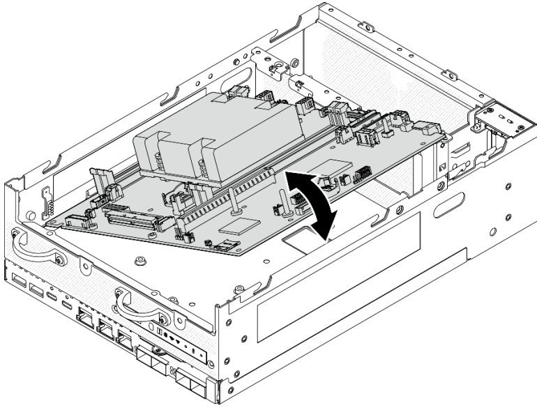
Figure 274. Installation de la carte mère
