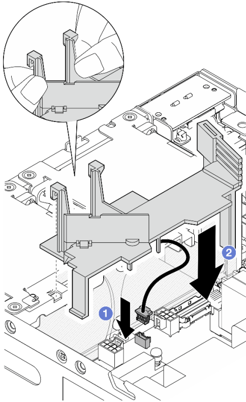
Figure 91. Installation de la grille d'aération
