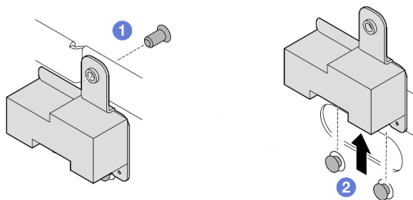
Figure 300. Retrait de l'obturateur SMA
