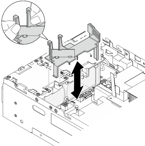
Figure 86. Retrait de la grille d'aération
