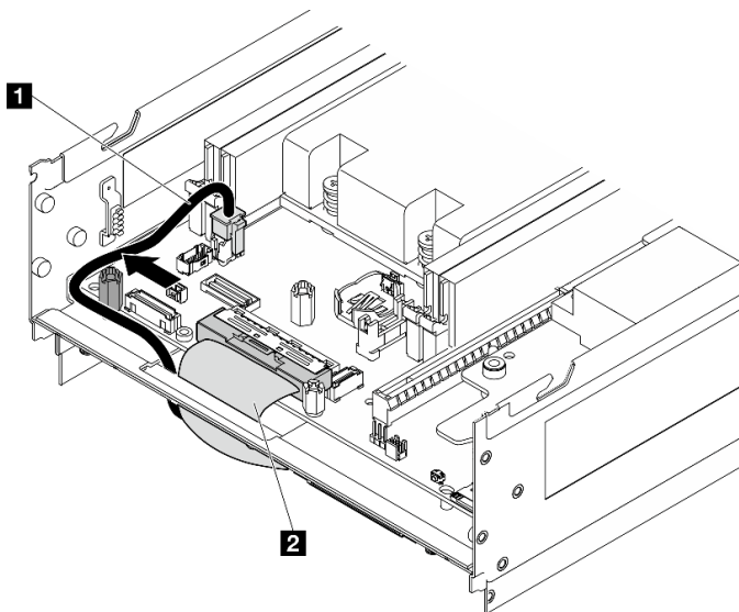
Figure 158. Cheminement des câbles de la carte d'E/S
