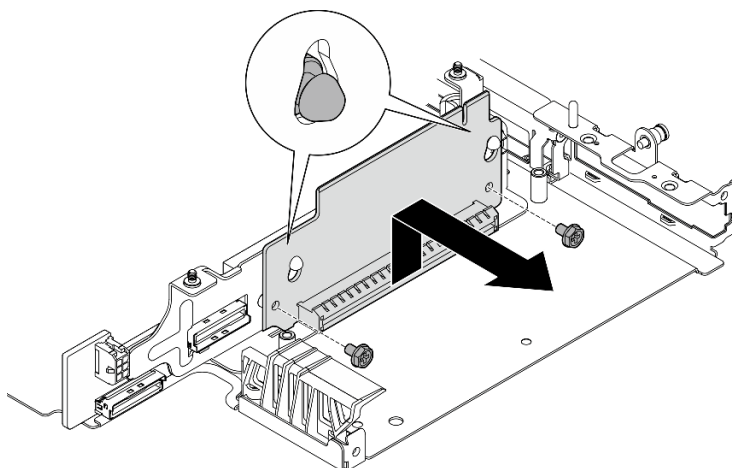
Figure 240. Retrait de la carte mezzanine
