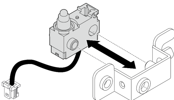
Figure 150. Séparation du commutateur d'intrusion du support
