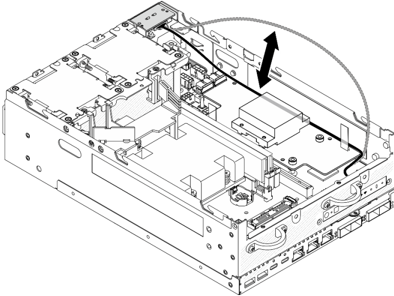
Figure 211. Placer le câble de signal
