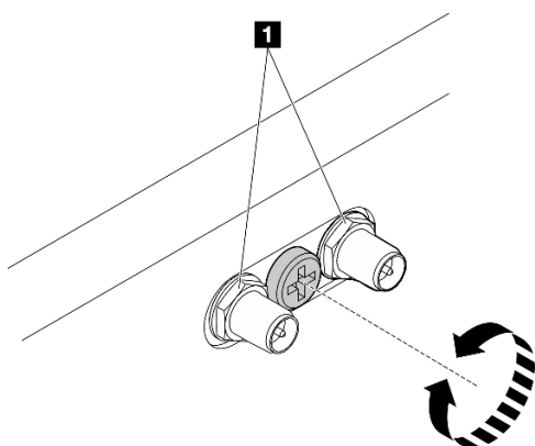
Figure 30. Raccourcissement des connecteurs SMA
