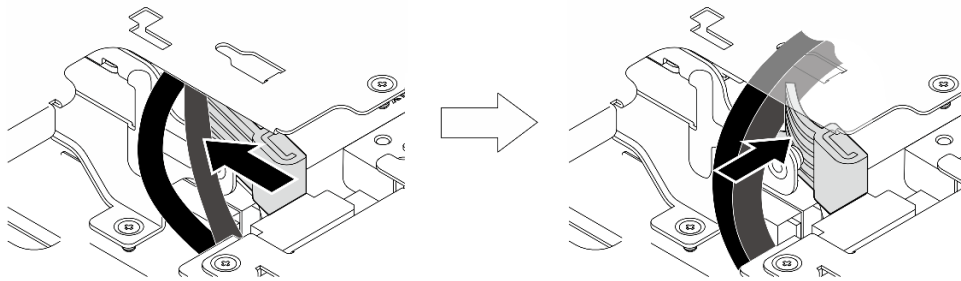
Figure 264. Cheminement des câbles
