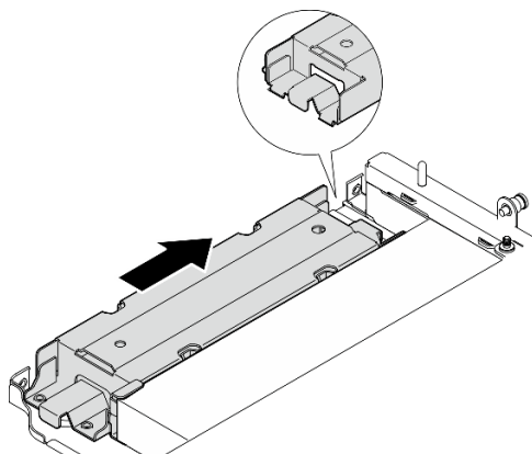
Figure 257. Installation du boîtier du module de géolocalisation
