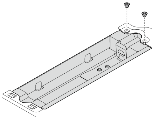
Figure 232. Retrait de l'boîtier du module de géolocalisation
