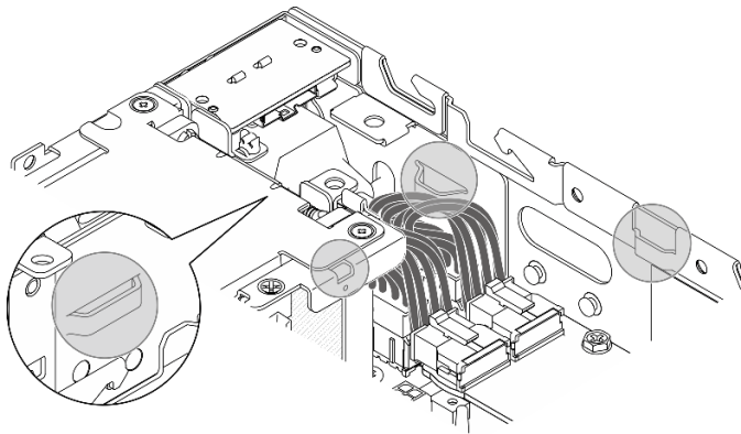
Figure 213. Les emplacements pour la grille d'aération PMB
