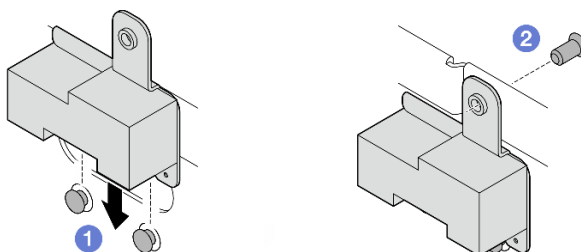
Figure 321. Installation de l'obturateur SMA
