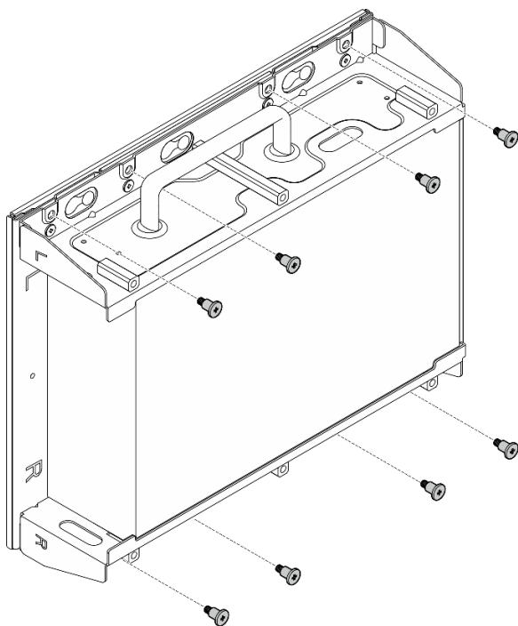
Figure 48. Installation du support de nœud
