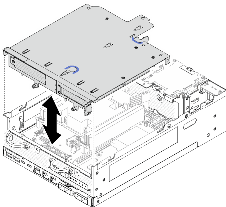
Figure 263. Abaisser l'assemblage de carte mezzanine
