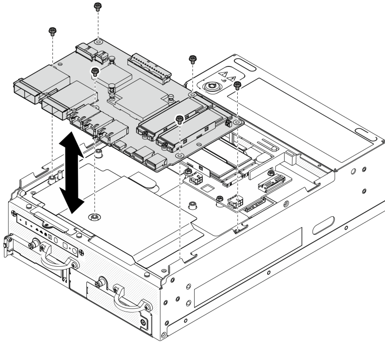
Figure 155. Retrait de la carte de module d'E/S
