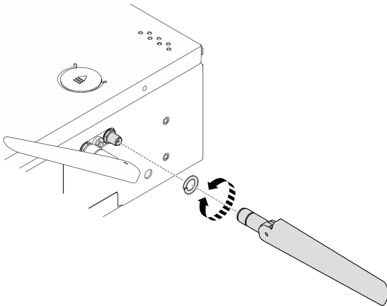
Figure 296. Retrait d'une antenne WLAN
