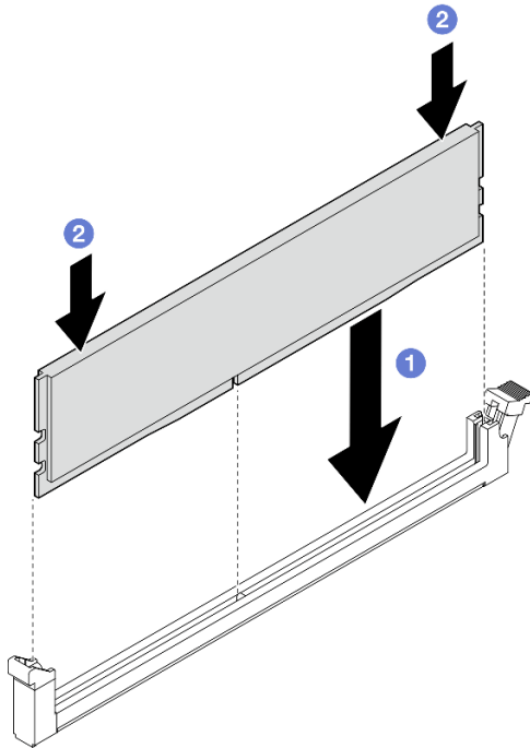
Figure 181. Installation d'un module de mémoire
