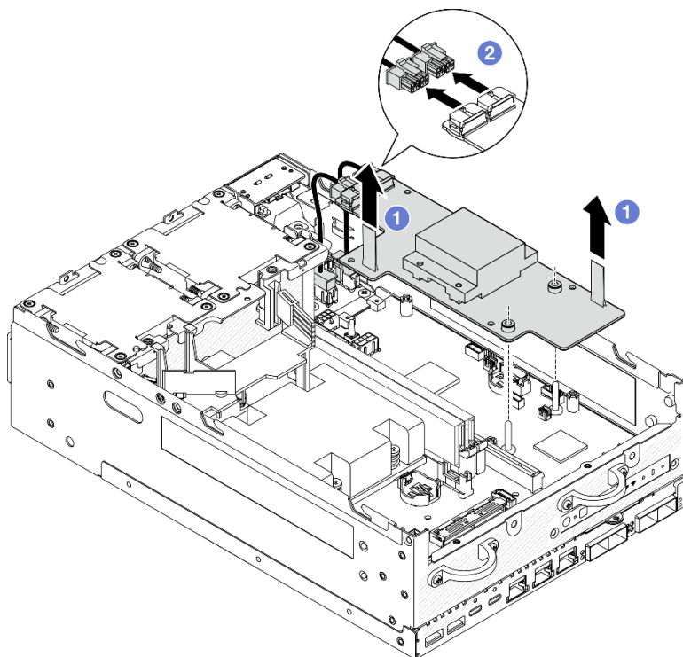
Figure 210. Retrait de la carte de module d'alimentation
