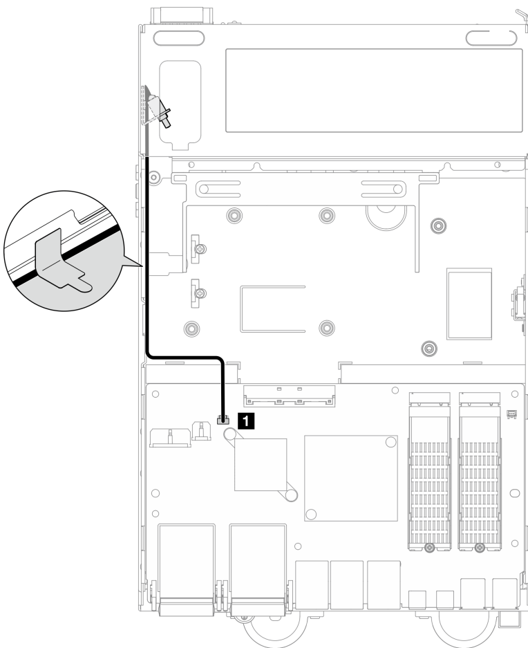
Figure 170. Cheminement des câbles du commutateur en position verrouillée
