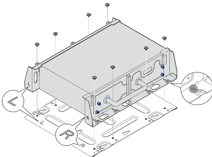
Figure 54. Retrait de la plaque inférieure
