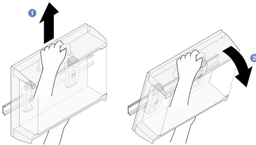
Figure 51. Retrait du manchon de nœud
