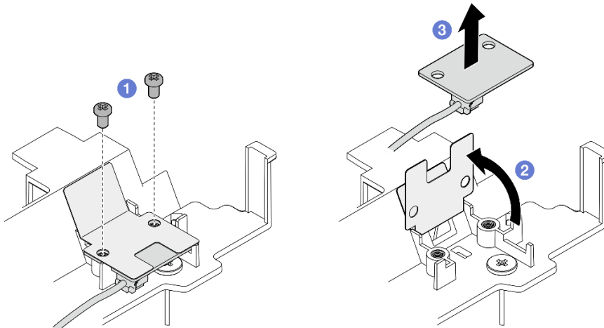
Figure 88. Retrait de la carte du capteur de ventilation
