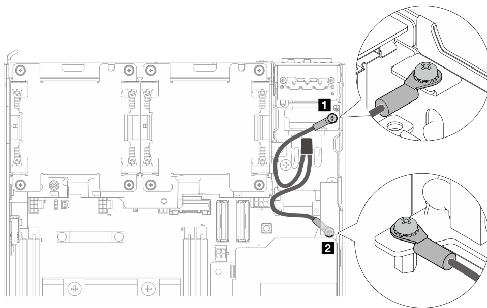
Figure 133. Déconnexion des câbles de mise à terre
