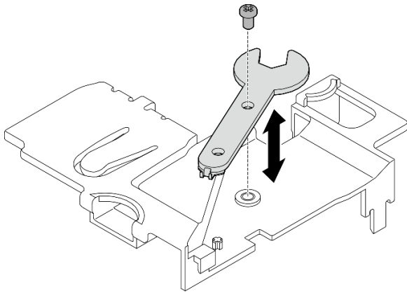
Figure 309. Rangement de la clé
