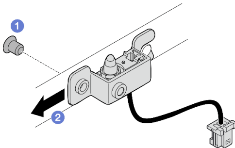
Figure 143. Retrait du commutateur d'intrusion avec câble
