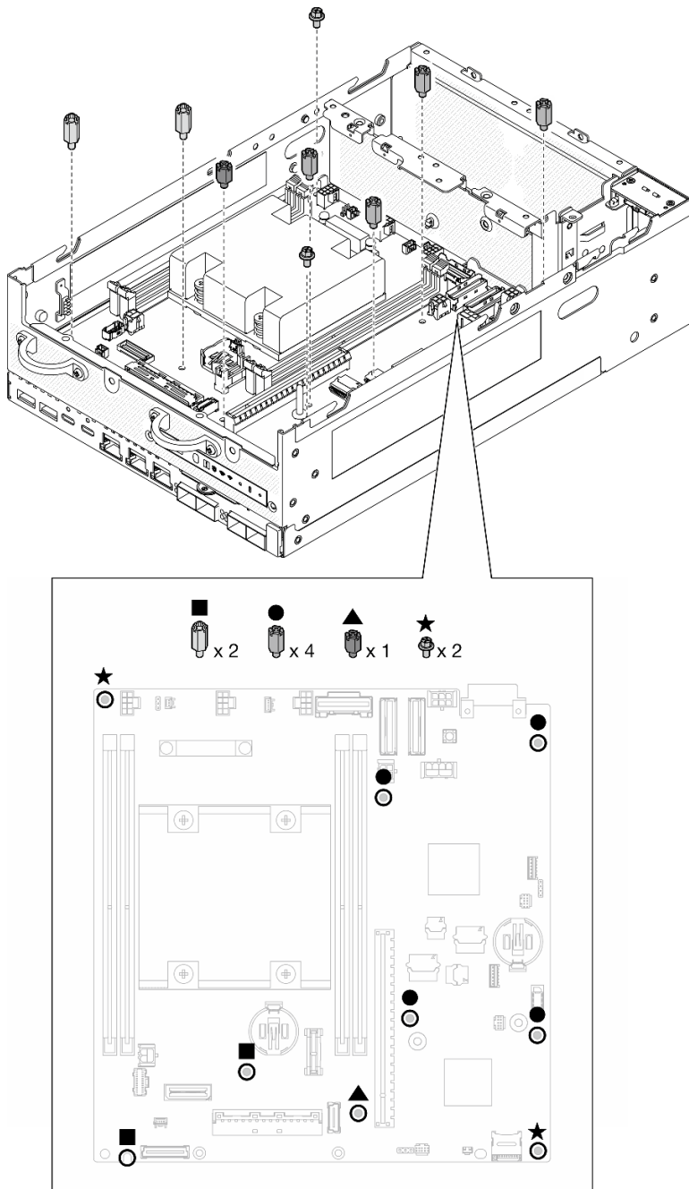
Figure 275. Les vis et les supports de la carte mère
