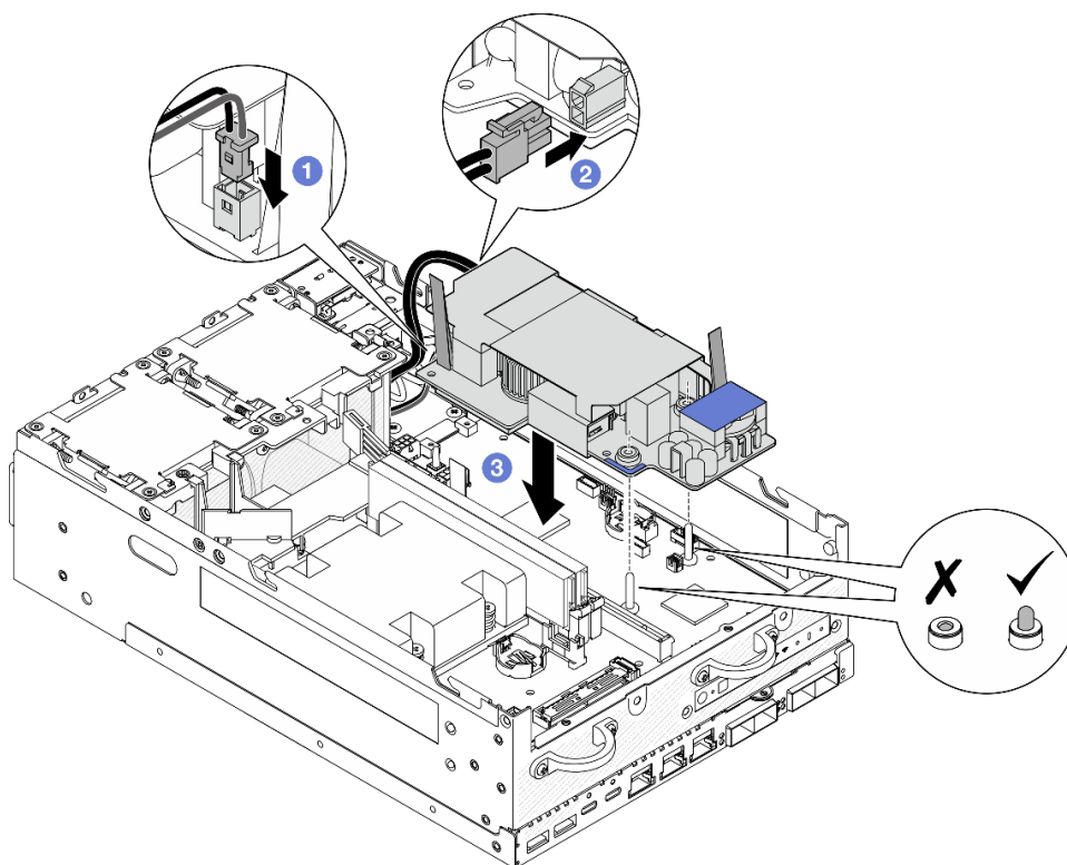
Figure 138. Installation du bloc d'alimentation interne
