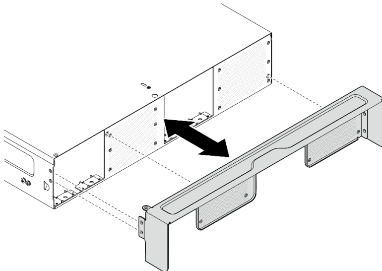
Figure 11. Retrait du support de transport
