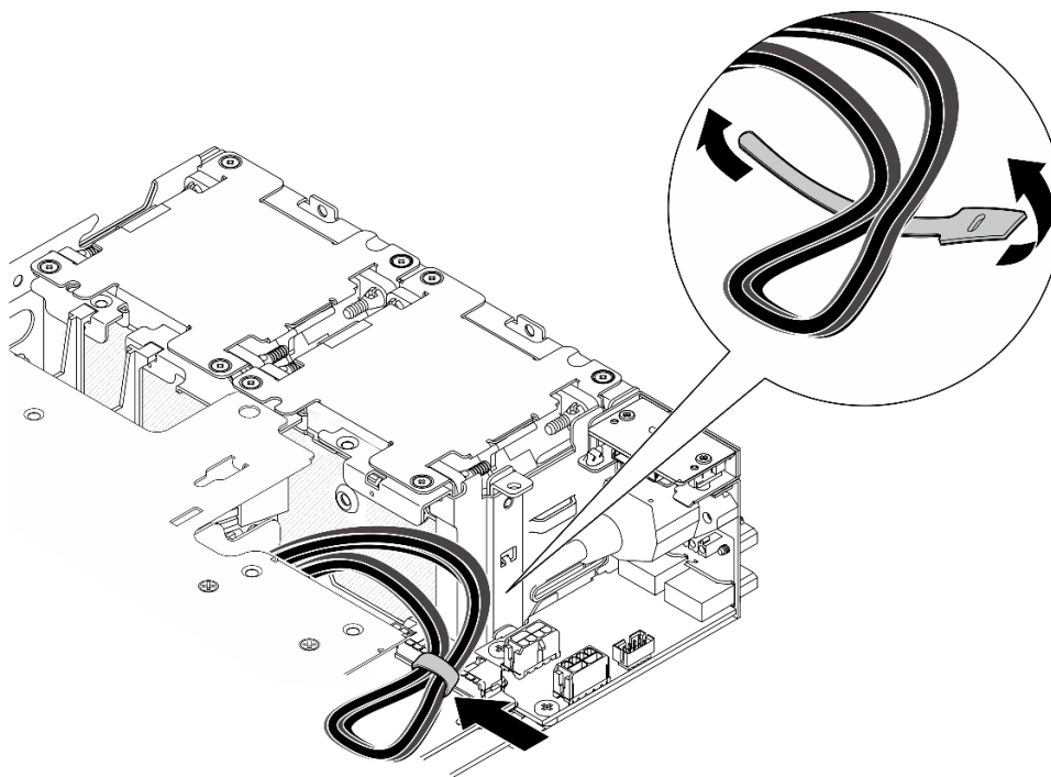
Figure 262. Cheminement des câbles pour l'assemblage de carte mezzanine
