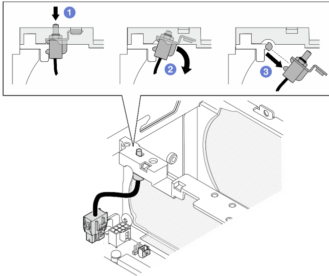
Figure 123. Retrait du commutateur d'orientation du ventilateur
