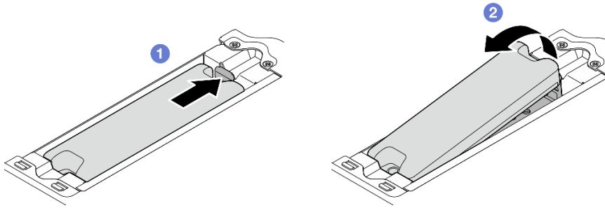
Figure 231. Retrait de l' module de géolocalisation
