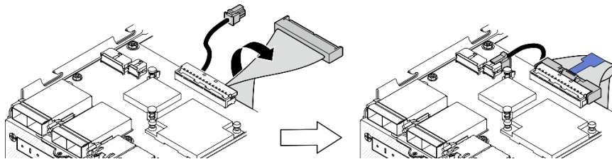
Figure 161. Connexion des câbles de la carte d'E/S
