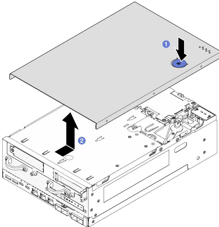
Figure 185. Retrait du carter supérieur
