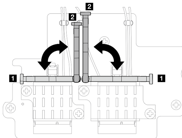
Figure 302. Faire pivoter le support de câble
