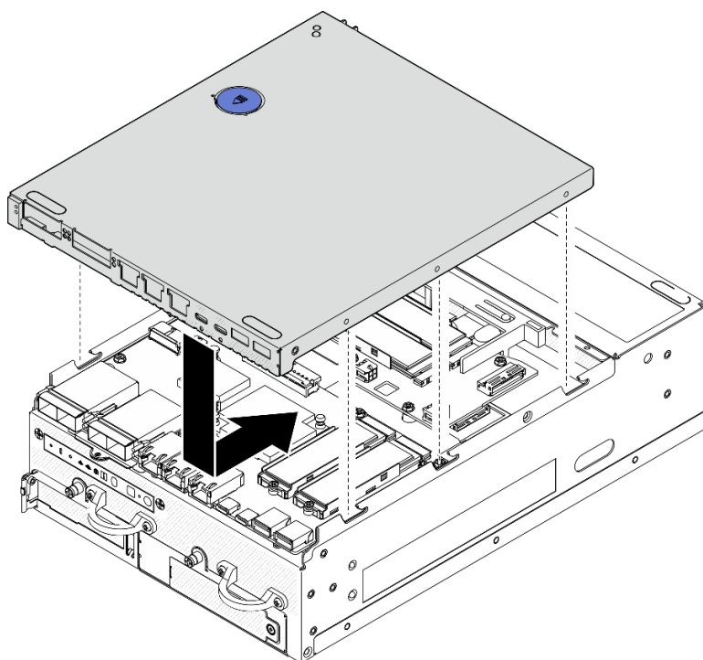
Figure 194. Installation du carter inférieur
