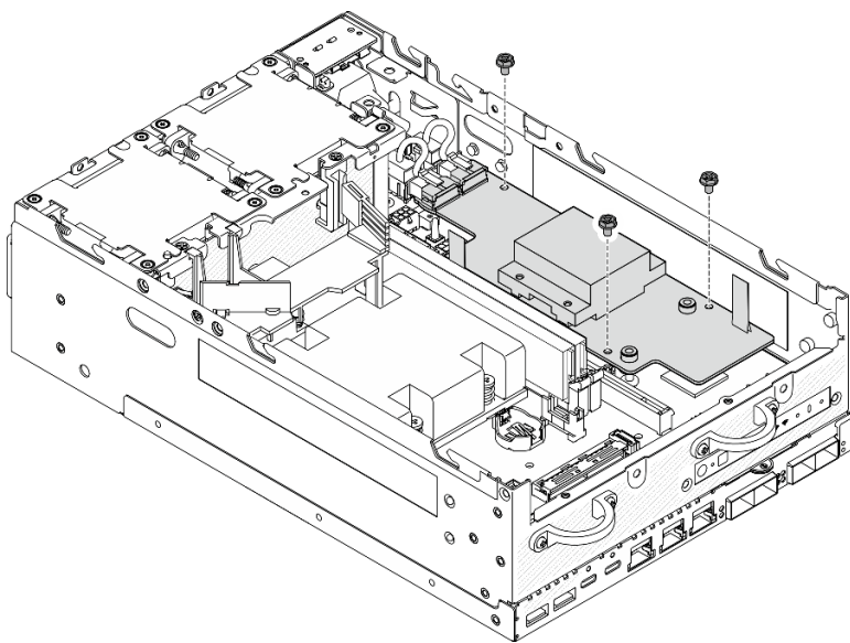
Figure 214. Fixation de la carte de module d'alimentation
