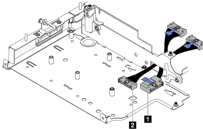
Figure 247. Câble de signal de l'adaptateur câblé M.2
