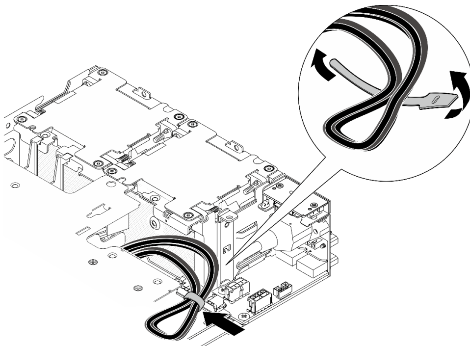
Figure 269. Cheminement des câbles pour l'assemblage de carte mezzanine
