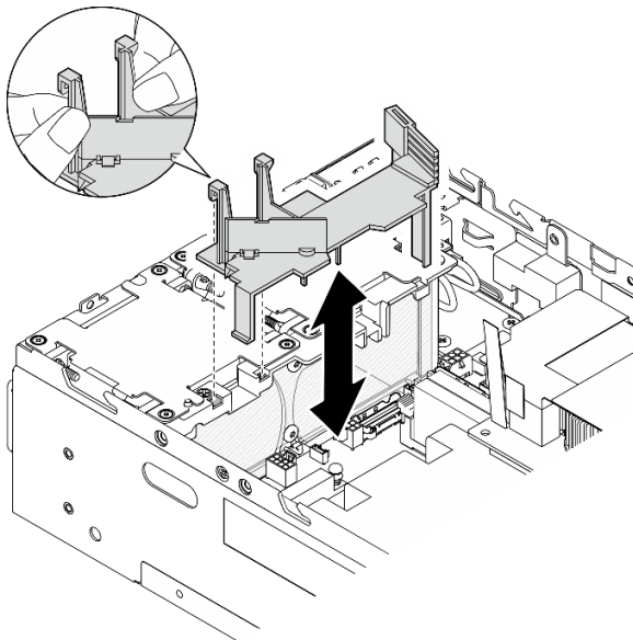
Figure 89. Installation de la grille d'aération
