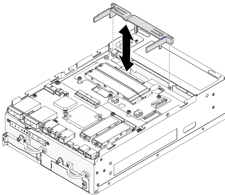
Figure 82. Retrait de la grille d'aération
