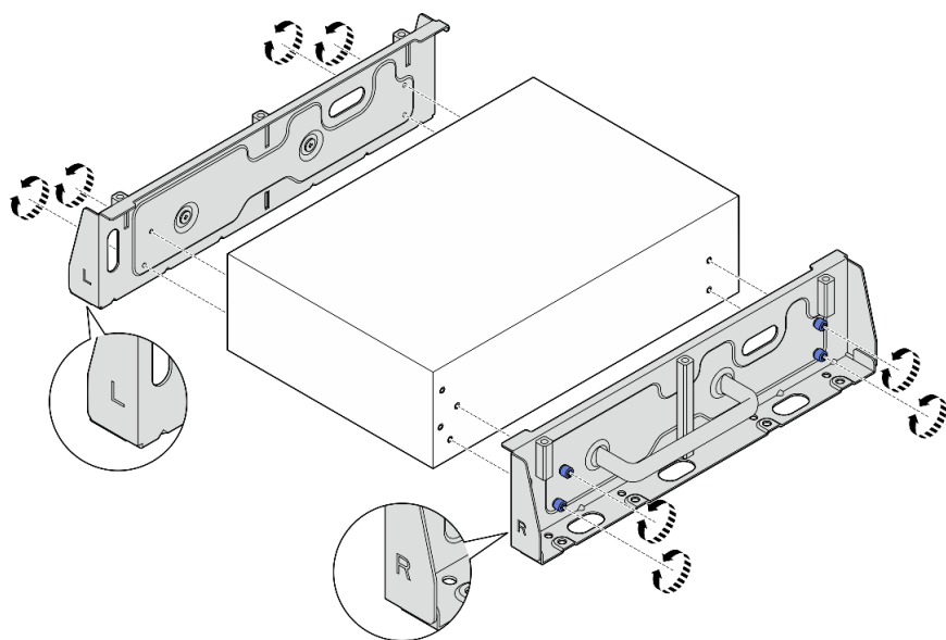
Figure 56. Desserrage des vis serrage à main pour retirer les supports latéraux
