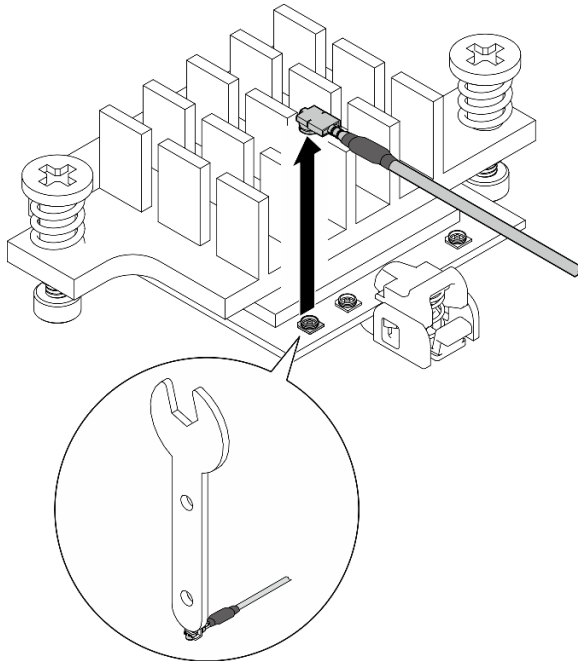
Figure 314. Déconnexion du câble
