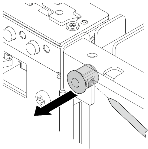
Figure 198. Retrait du câble du voyant d'état PMB
