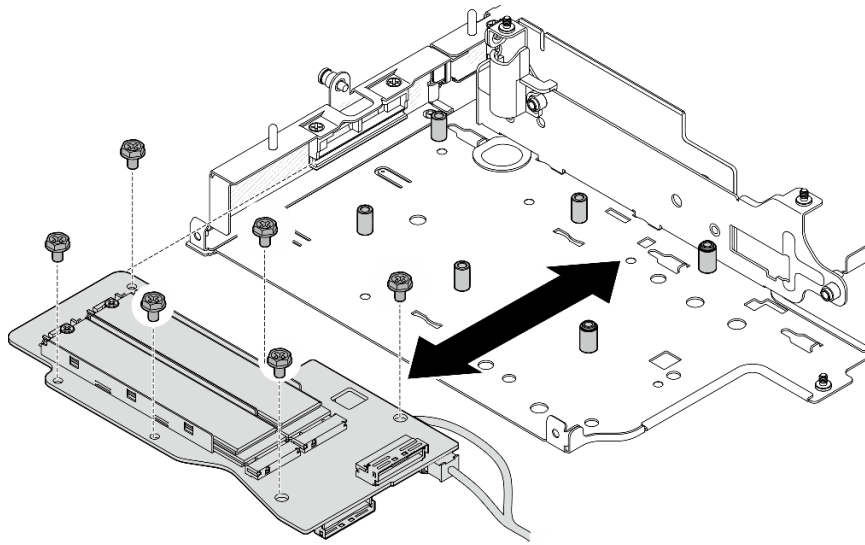
Figure 225. Retrait de l'adaptateur M.2 câblé
