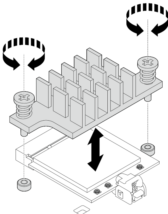
Figure 281. Retrait du dissipateur thermique et du module WLAN/Bluetooth
