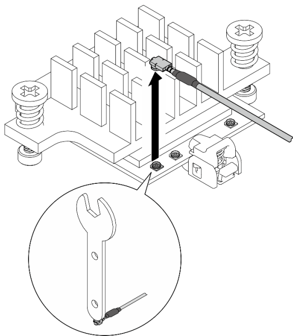
Figure 280. Déconnexion du câble
