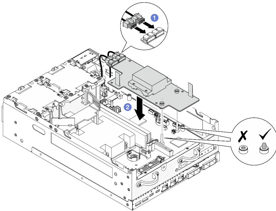
Figure 212. Installation de la carte de module d'alimentation
