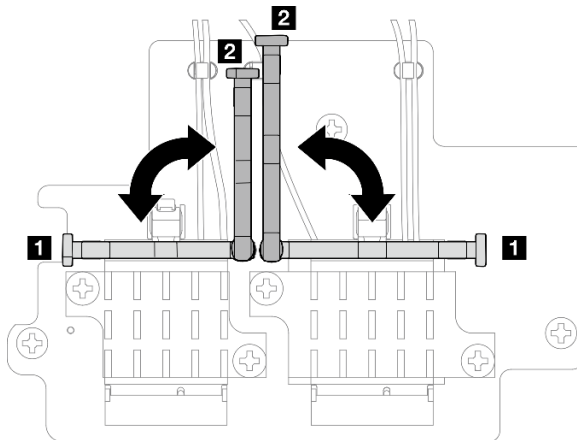
Figure 292. Faire pivoter le support de câble
