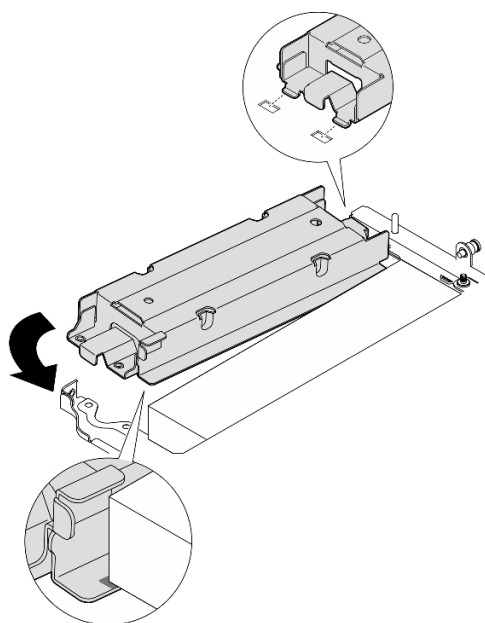
Figure 256. Installation du boîtier du module de géolocalisation
