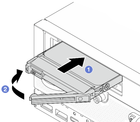
Figure 79. Installation d'une unité 7 mm
