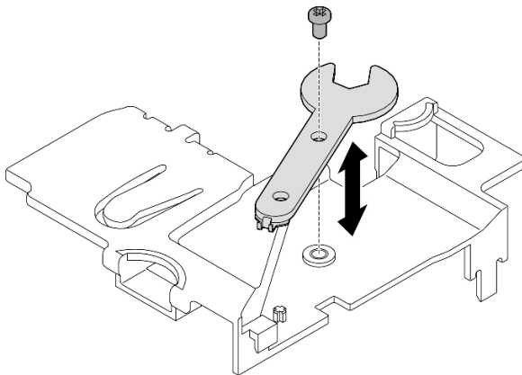
Figure 320. Rangement de la clé
