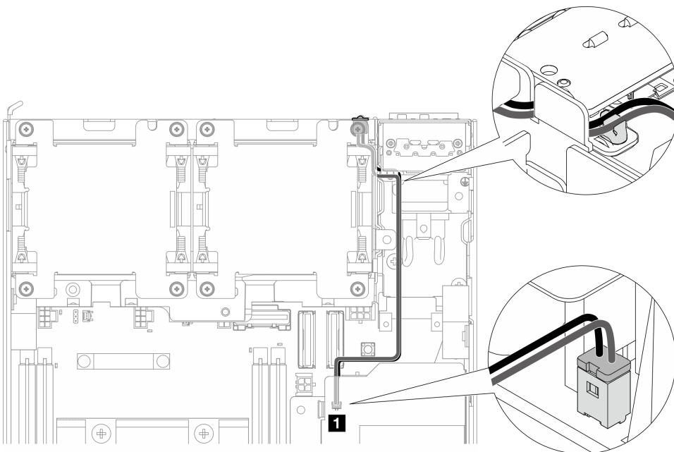
Figure 201. Câble du voyant d'état du PMB se connectant au bloc d'alimentation interne (PMB CA)
