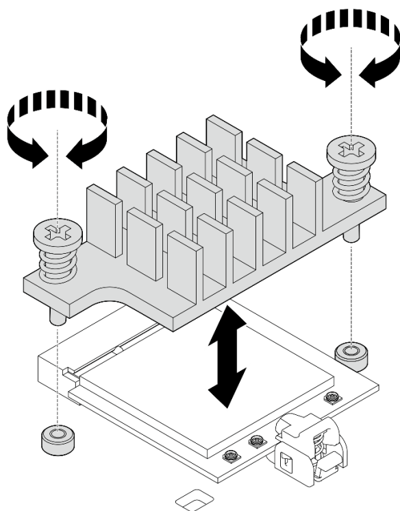
Figure 289. Installation du dissipateur thermique du module WLAN/Bluetooth
