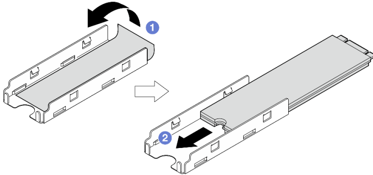
Figure 174. Installation de l'unité M.2
