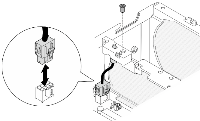
Figure 122. Retrait du commutateur d'orientation du ventilateur
