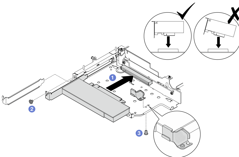
Figure 251. Installation de l'adaptateur PCIe
