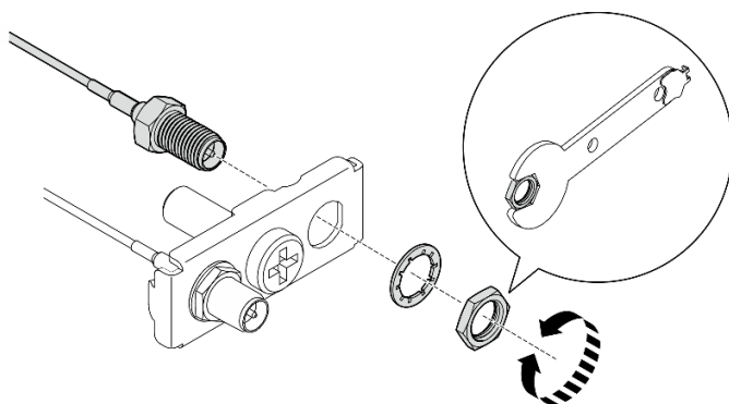
Figure 325. Fixation des câbles au support
