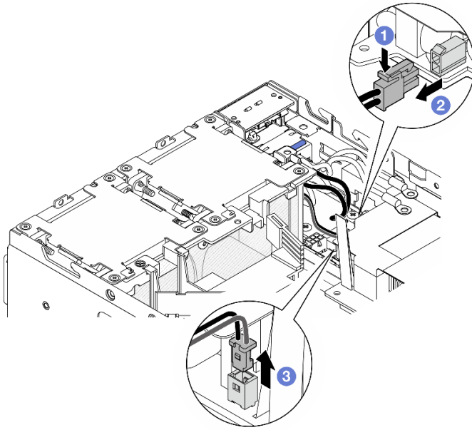
Figure 134. Déconnexion des câbles
