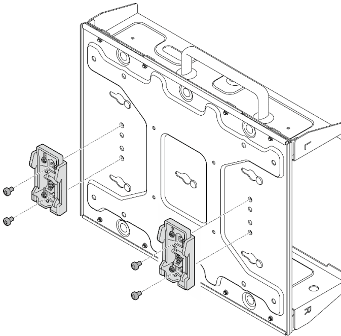
Figure 63. Installation des clips pour la glissière DIN
