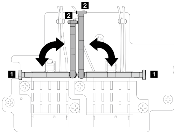
Figure 304. Faire pivoter le support de câble
