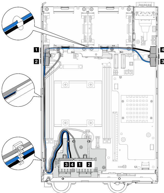
Figure 327. Cheminement de câble pour les assemblages SMA
