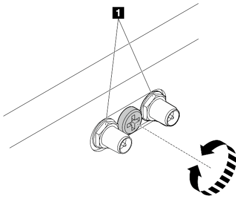
Figure 19. Raccourcissement des connecteurs SMA
