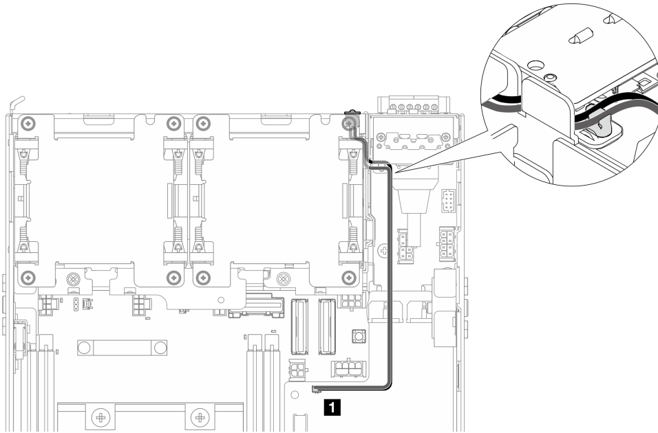
Figure 208. Câble de la LED de la PMB
