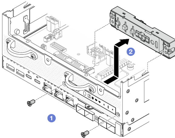
Figure 130. Retrait du panneau opérateur avant
