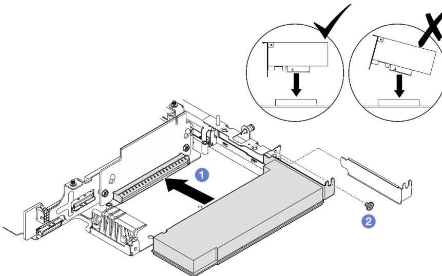
Figure 245. Installation de l'adaptateur PCIe
