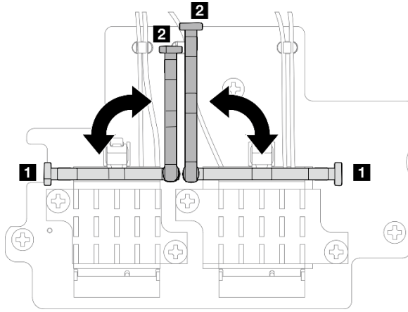
Figure 95. Faire pivoter le support de câble
