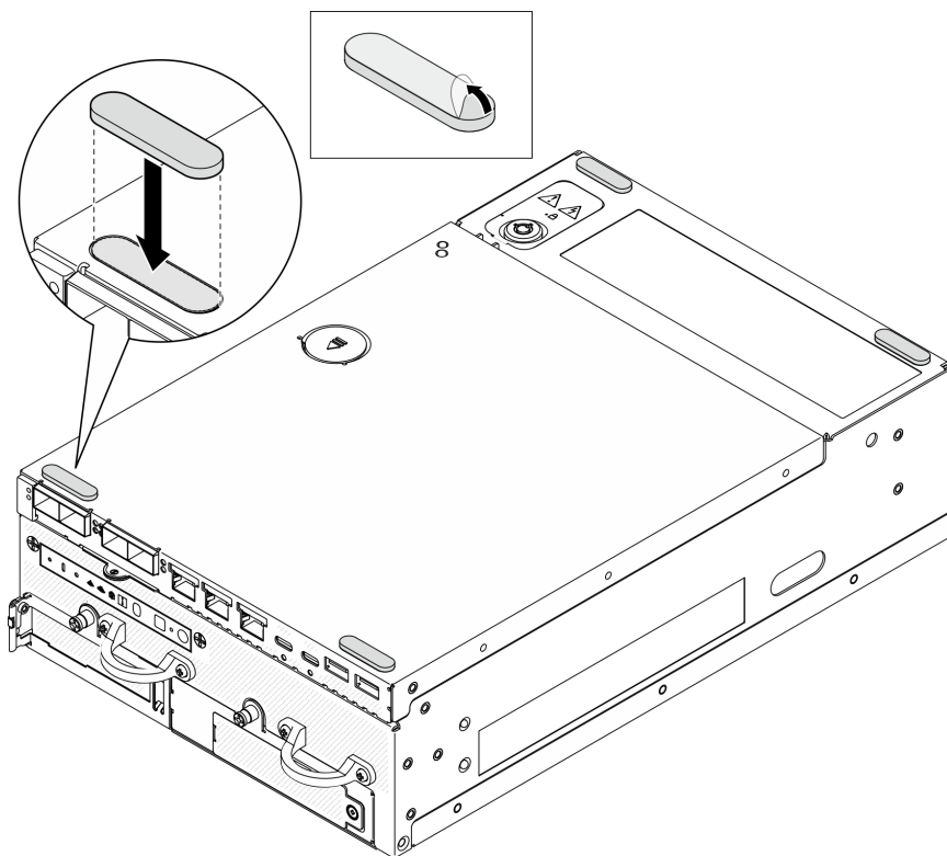
Figure 271. Installation des pieds en caoutchouc
