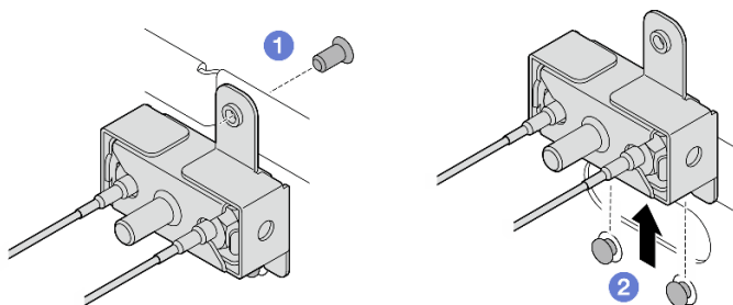
Figure 317. Retrait de l'assemblage SMA
