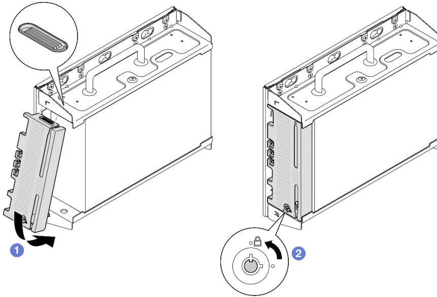
Figure 65. Installation du panneau de sécurité
