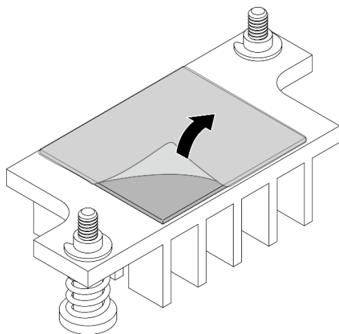
Figure 288. Retrait du film du tampon thermique
