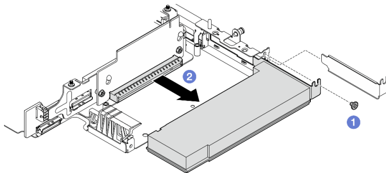
Figure 239. Retrait de l'adaptateur PCIe
