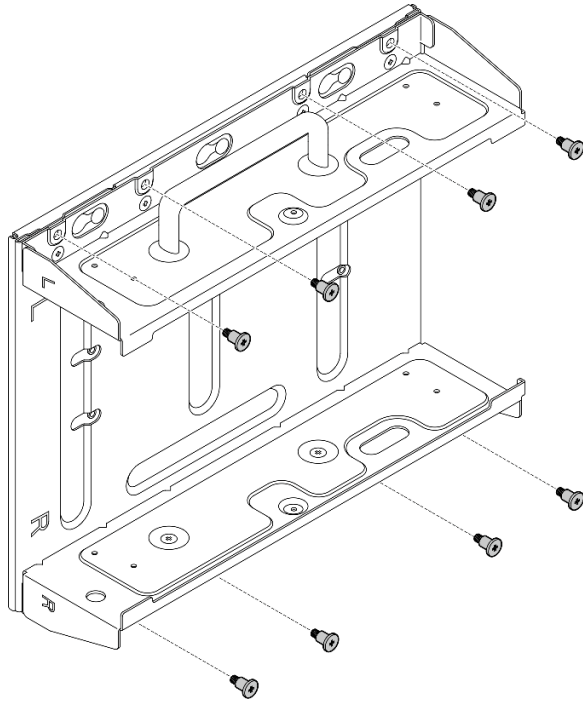
Figure 27. Retrait du support du nœud
