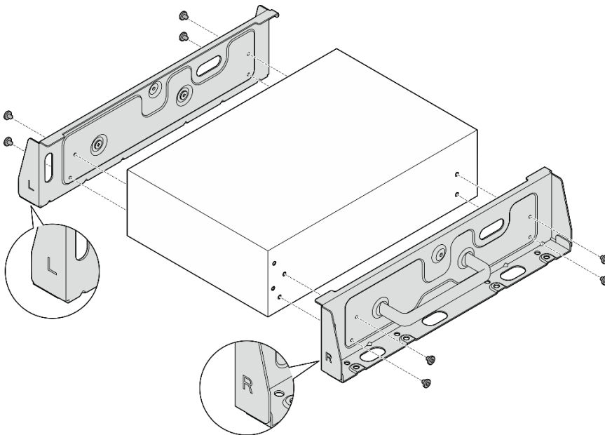
Figure 40. Installation des supports latéraux avec des vis
