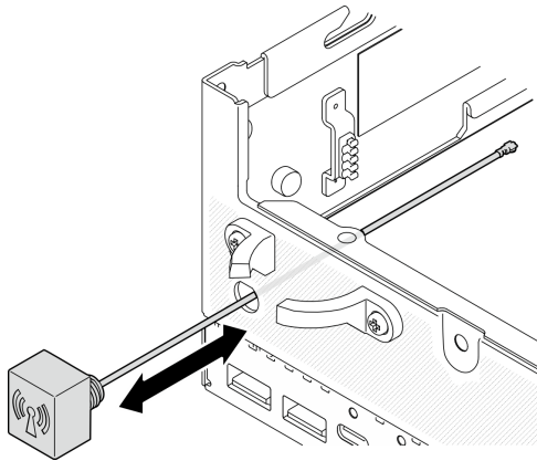
Figure 100. Retrait de l'antenne Bluetooth
