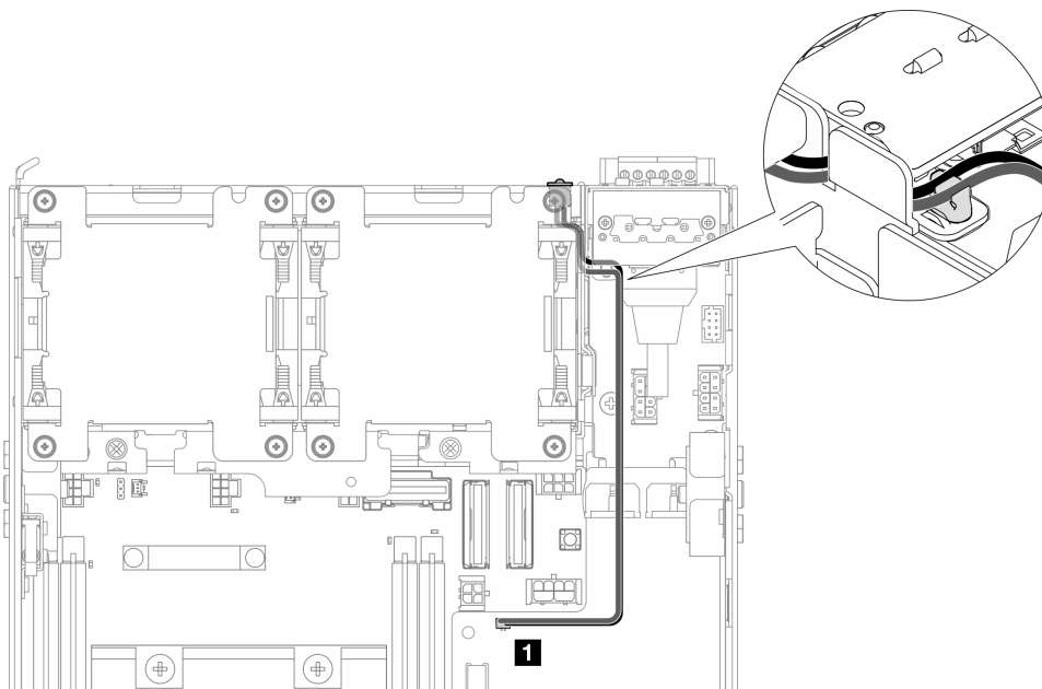
Figure 215. Câble de la LED de la PMB
