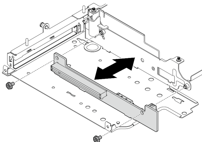
Figure 228. Retrait de la carte mezzanine
