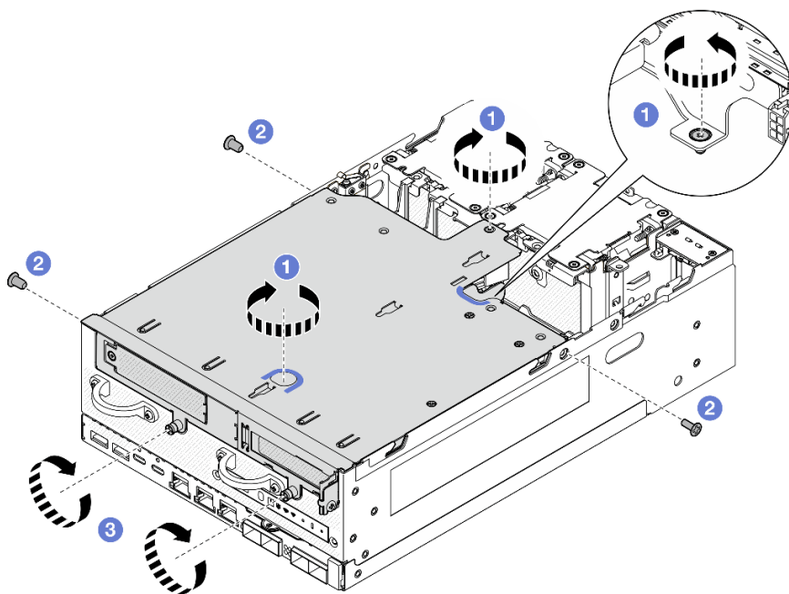
Figure 261. Fixer l'assemblage de carte mezzanine
