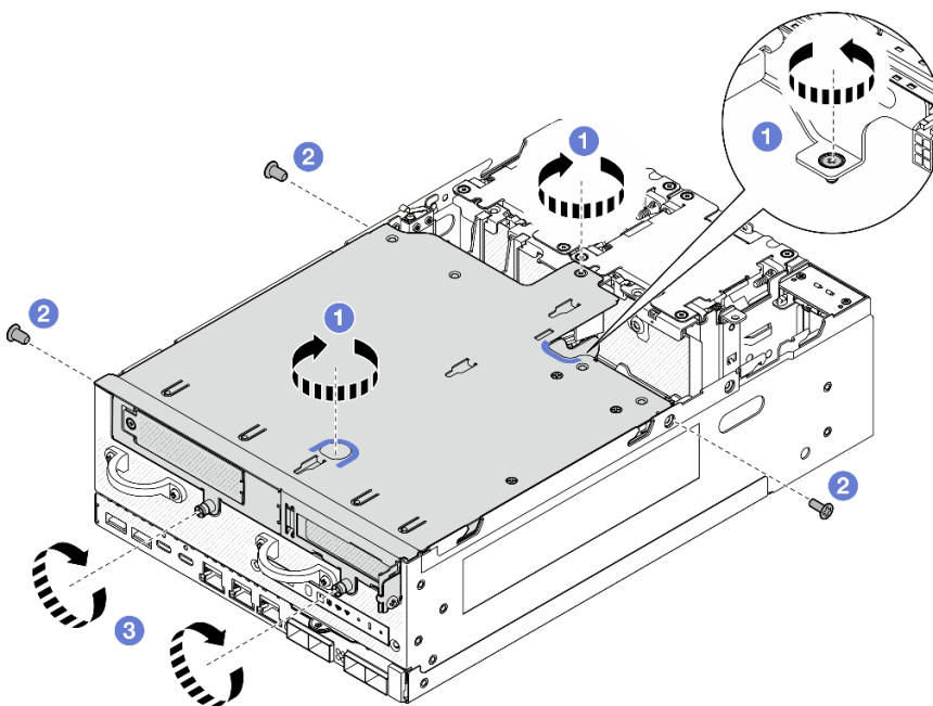
Figure 268. Fixer l'assemblage de carte mezzanine
