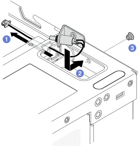
Figure 169. Installation du commutateur en position verrouillée avec câble
