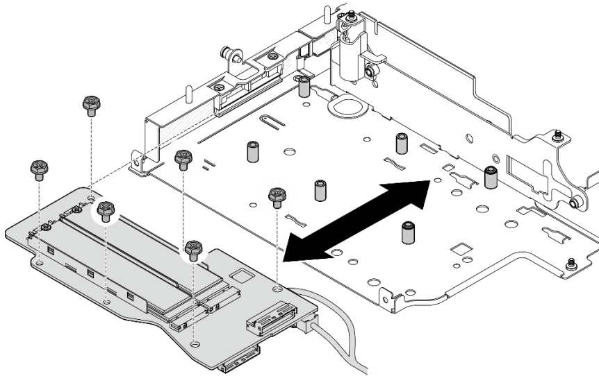
Figure 248. Installation de l'adaptateur M.2
