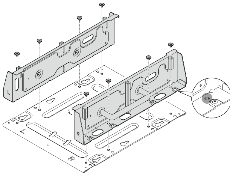
Figure 38. Démonter le support du nœud
