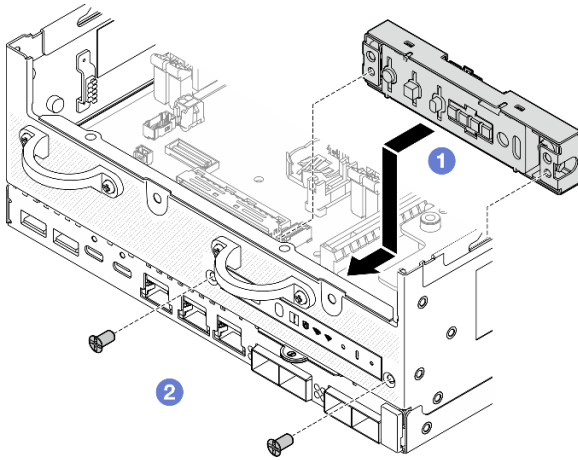
Figure 131. Installation du panneau opérateur avant
