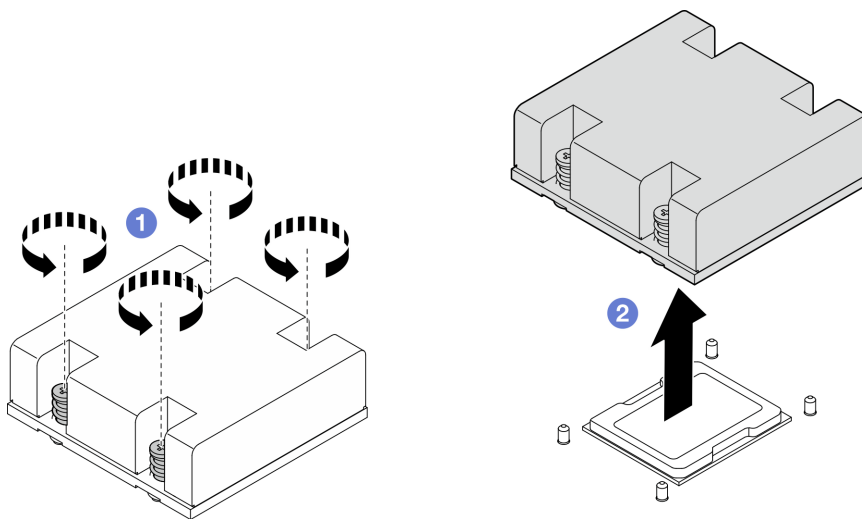
Figure 217. Retrait du dissipateur thermique de processeur
