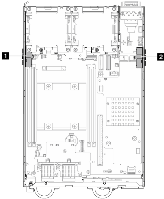
Figure 297. Lieux d'assemblages SMA
