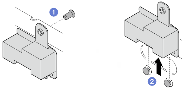
Figure 311. Retrait de l'obturateur SMA
