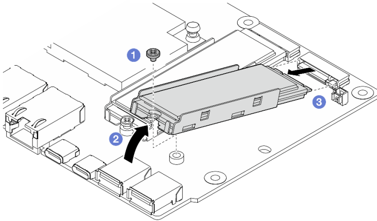
Figure 154. Retrait d'une unité M.2
