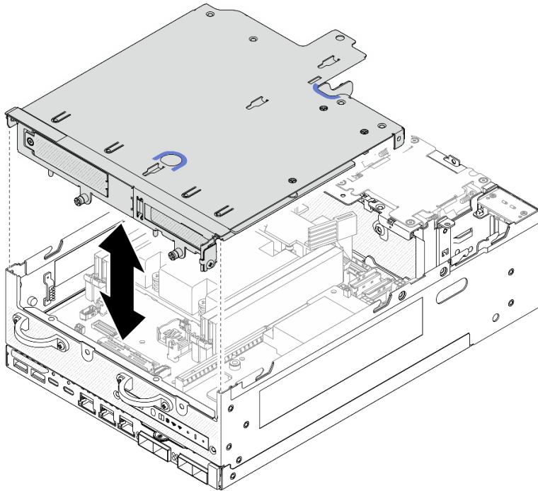
Figure 223. Soulever l'assemblage de carte mezzanine
