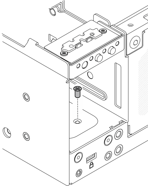
Figure 172. Fixation de la vis
