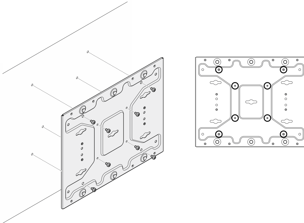
Figure 29. Retrait de la plaque de montage murale
