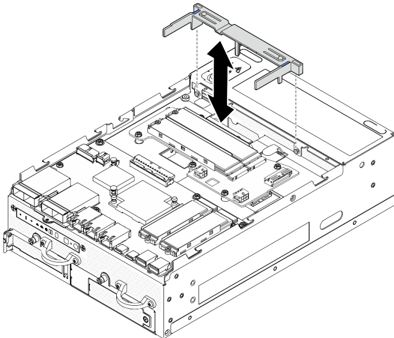
Figure 83. Installation de la grille d'aération
