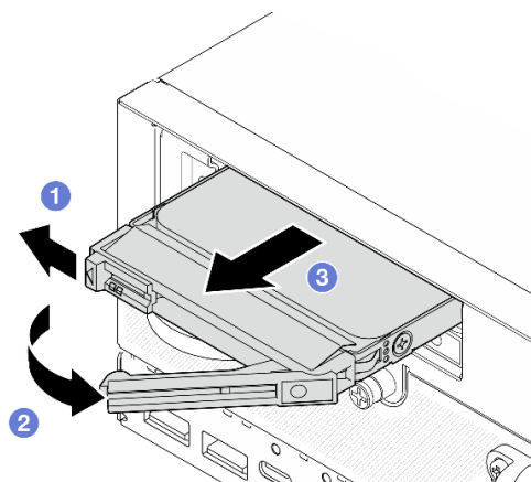
Figure 77. Retrait d'une unité 7 mm
