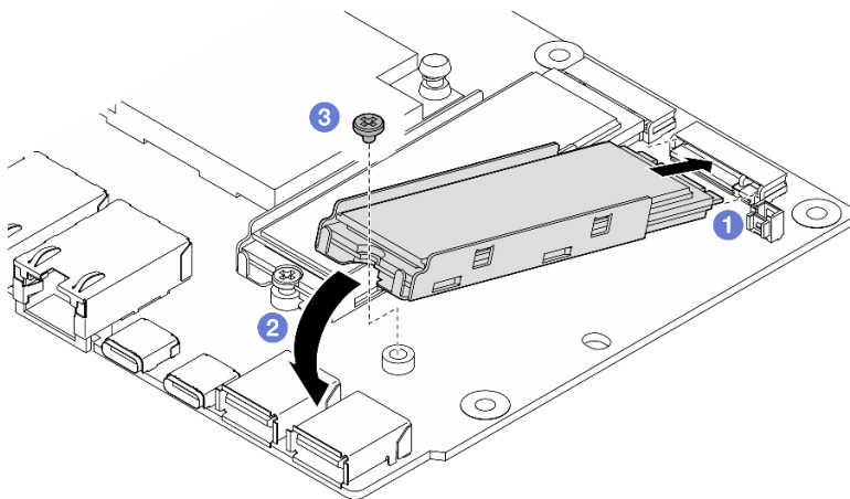
Figure 162. Installation d'une unité M.2
