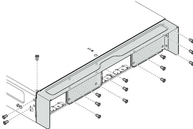
Figure 10. Desserer les vis
