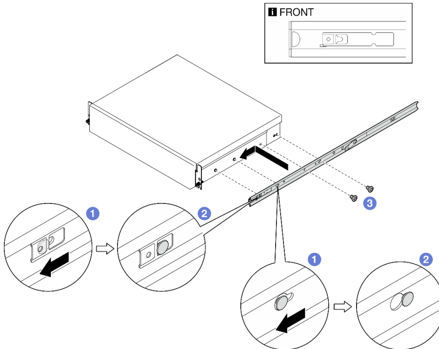
Figure 16. Installation de la glissière interne
