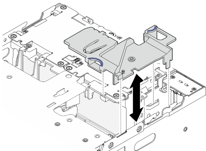
Figure 84. Retrait de la grille d'aération
