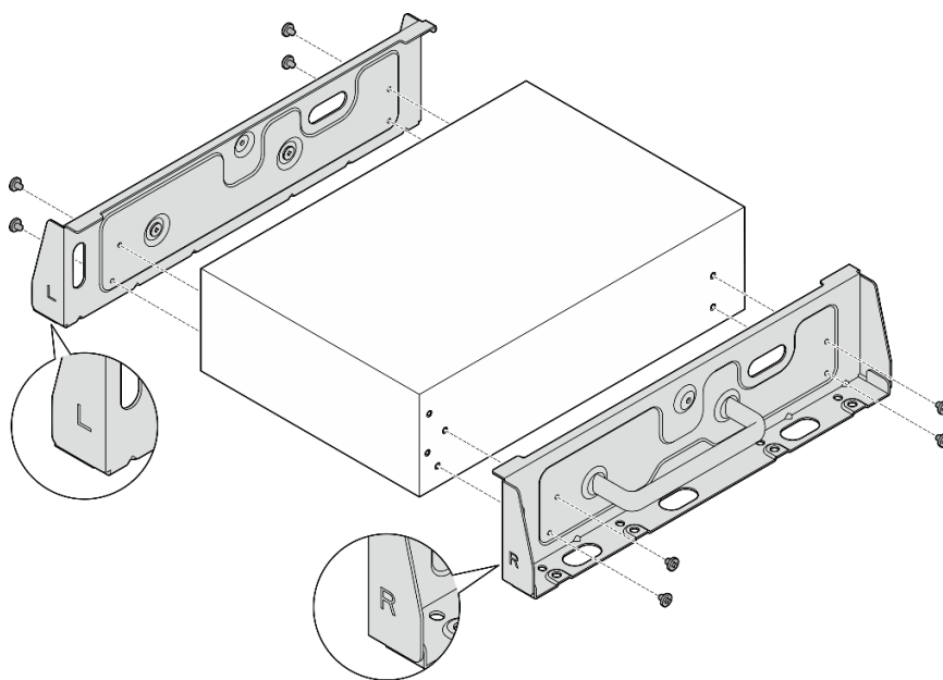
Figure 32. Desserrage des vis pour retirer les supports latéraux
