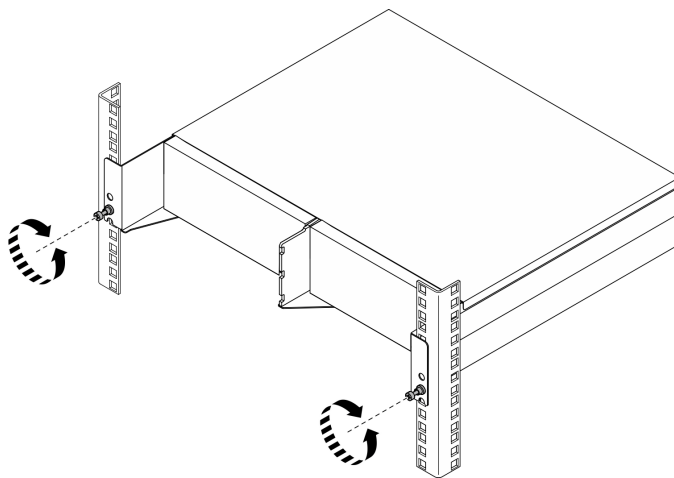
Figure 18. Fixation du boîtier dans l'armoire
