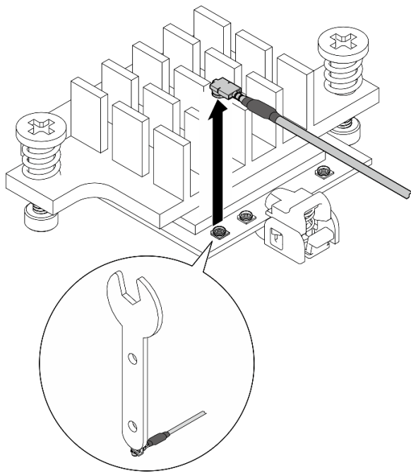
Figure 303. Déconnexion du câble
