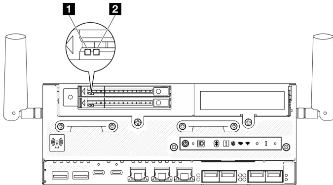
Figure 347. Voyants d'unité
