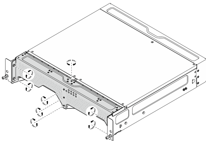
Figure 66. Desserrer les vis
