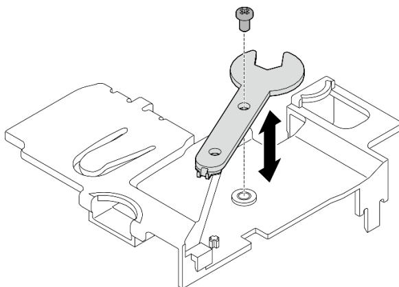
Figure 335. Rangement de la clé
