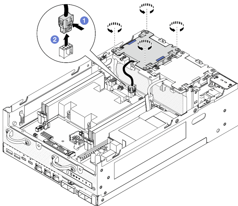
Figure 126. Retrait du module de ventilation
