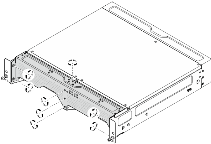
Figure 2. Desserer les vis
