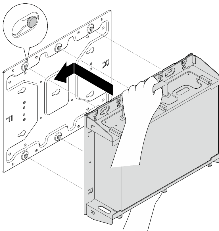
Figure 47. Installation du support de nœud
