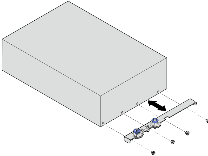
Figure 6. Retrait du support du boîtier
