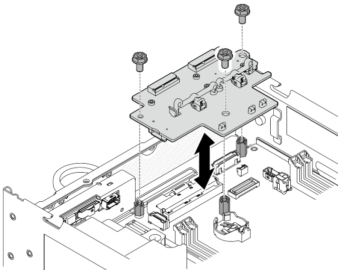
Figure 284. Installation de l'adaptateur sans fil
