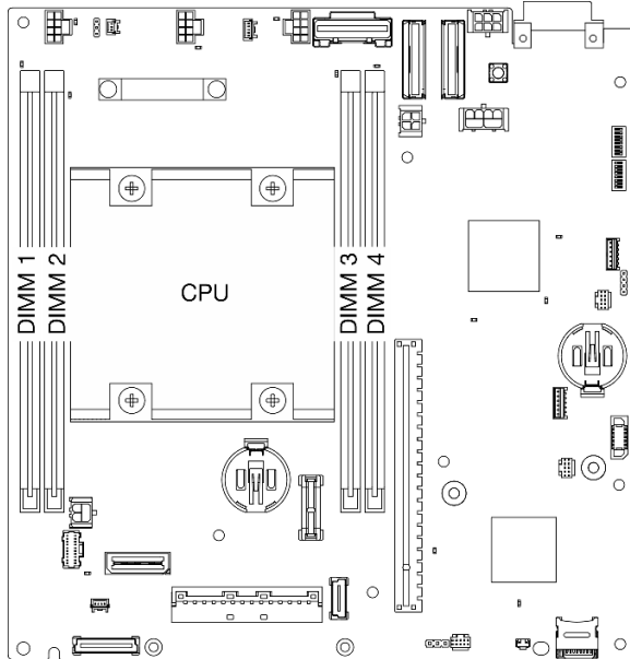
Figure 176. Disposition des modules de mémoire et des processeurs
