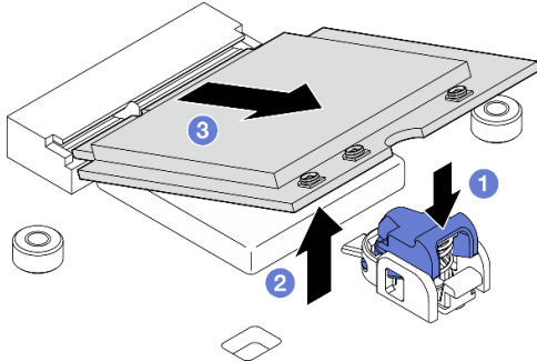
Figure 282. Retrait du module WLAN/Bluetooth
