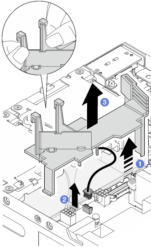
Figure 87. Retrait de la grille d'aération
