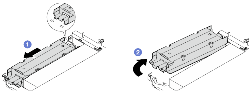
Figure 233. Retrait de l'boîtier du module de géolocalisation
