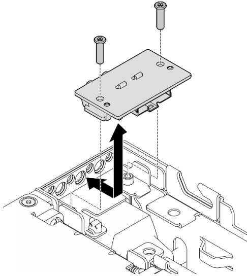
Figure 220. Retrait du panneau opérateur arrière
