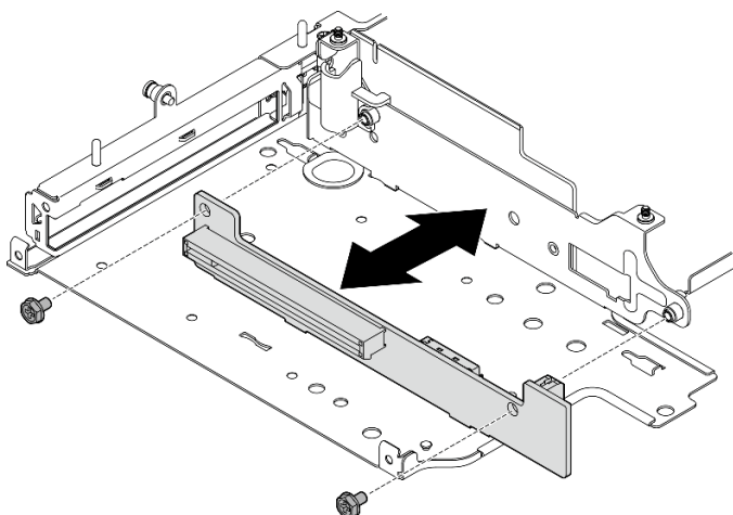
Figure 254. Installation de la carte mezzanine
