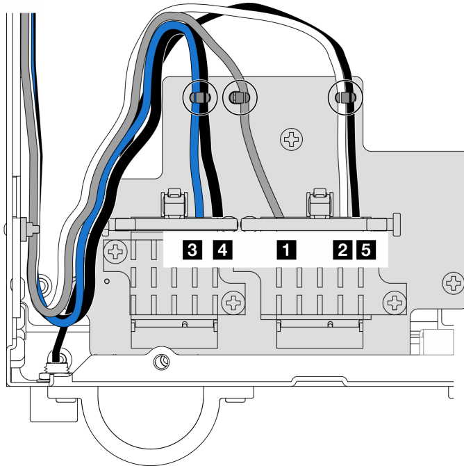
Figure 330. Cheminement des câbles pour l'adaptateur sans fil
