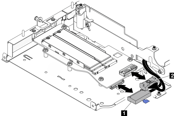
Figure 224. Débranchement du câble de signal
