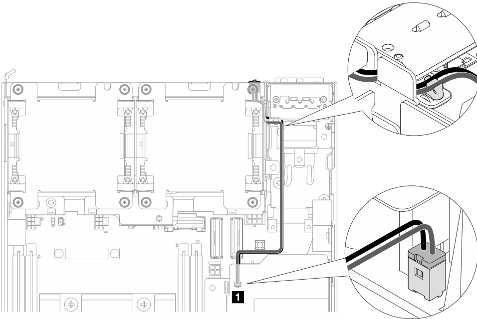
Figure 197. Câble du voyant d'état du PMB se connectant au bloc d'alimentation interne (PMB CA)
