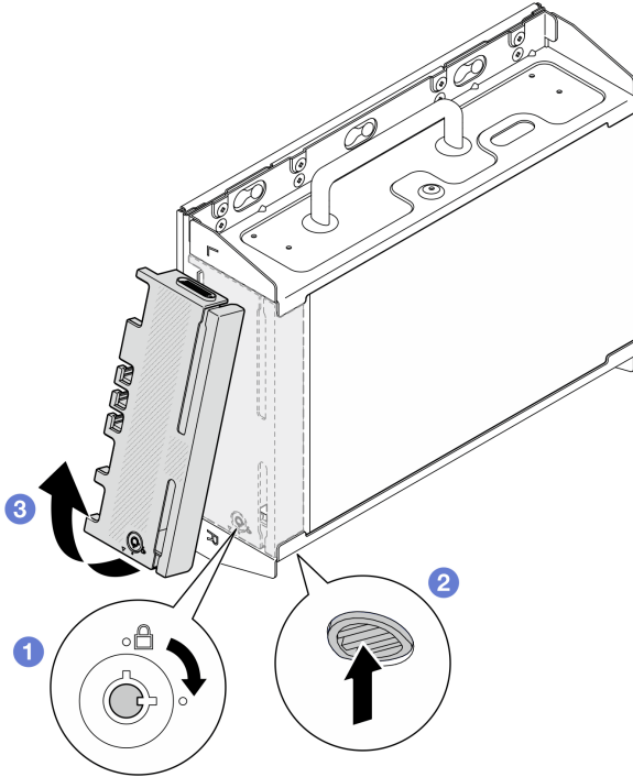
Figure 50. Retrait du panneau de sécurité
