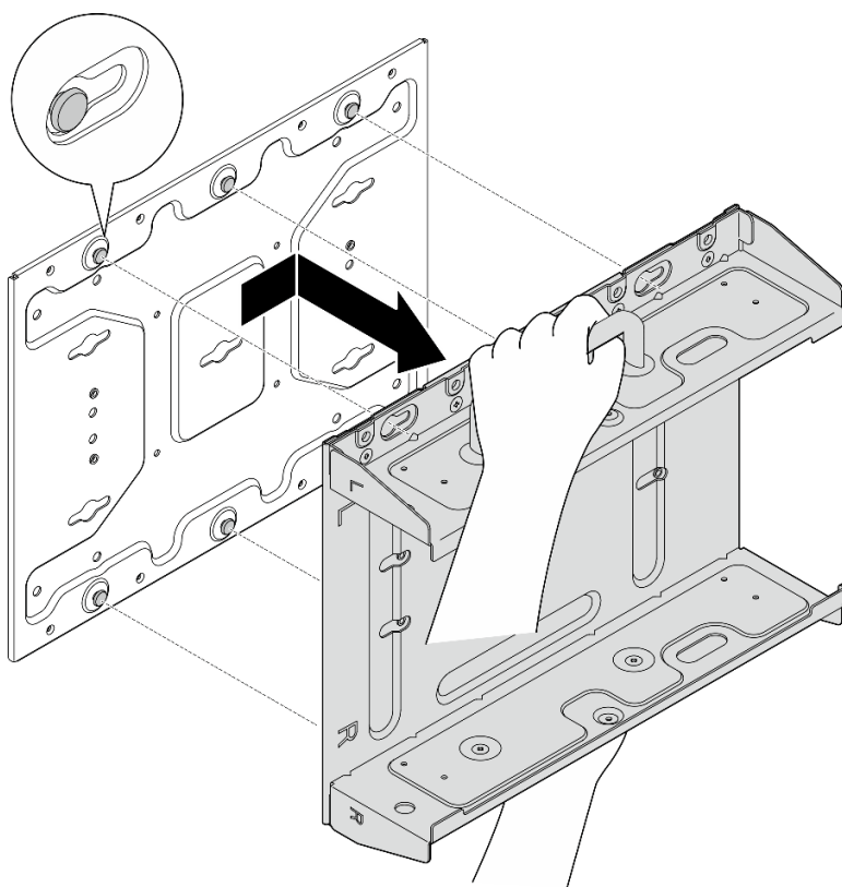
Figure 28. Retrait du support du nœud
