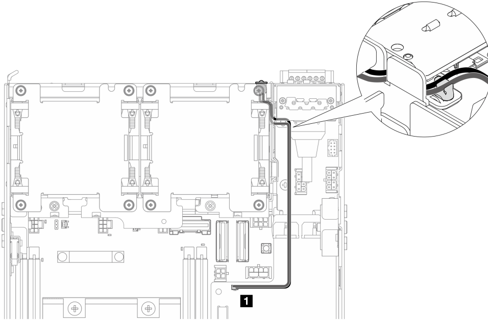
Figure 196. Câble du voyant d'état du PMB se connectant à la carte du module d'alimentation CC (PMB CC)
