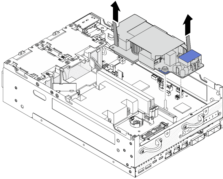
Figure 136. Retrait du bloc d'alimentation interne
