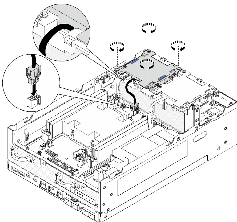
Figure 129. Installation du module de ventilation
