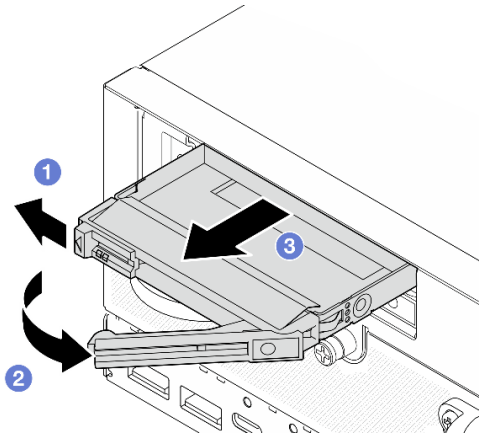
Figure 78. Retrait d'un obturateur d'unité
