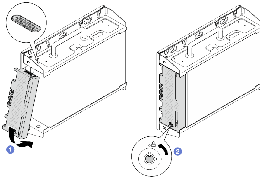
Figure 49. Installation du panneau de sécurité
