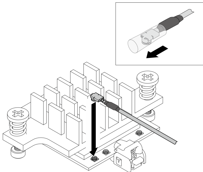
Figure 107. Connexion du câble
