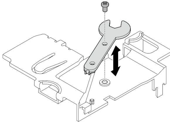
Figure 322. Désengagement de la clé
