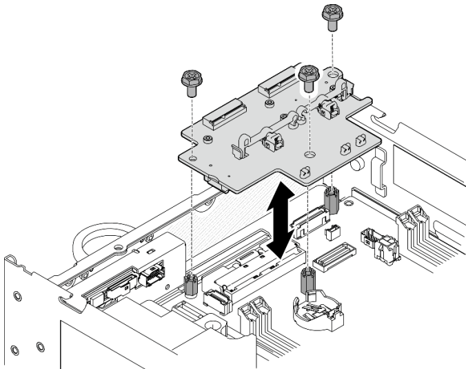
Figure 283. Retrait de l'adaptateur sans fil
