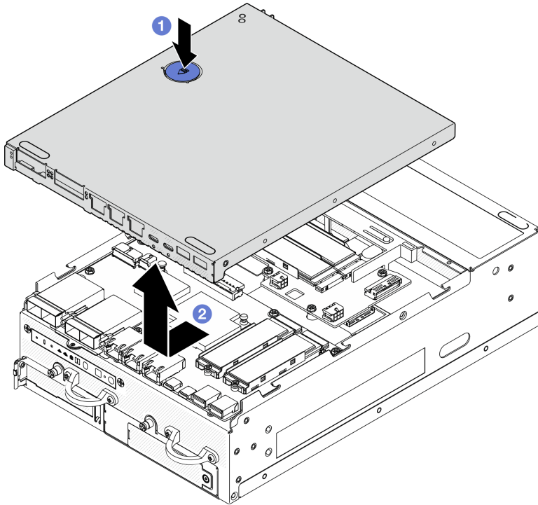
Figure 191. Retrait du carter inférieur
