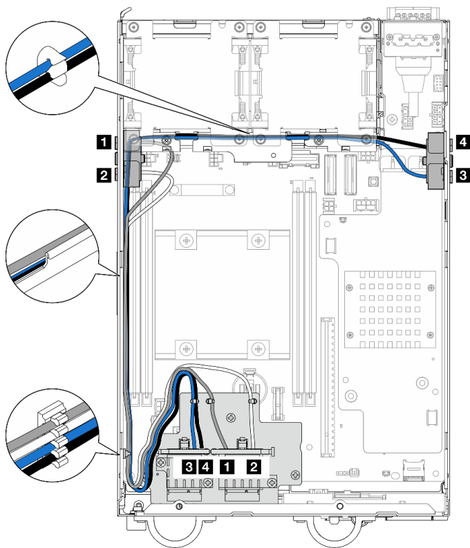
Figure 342. Cheminement du câble d'antenne WLAN
