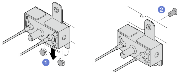
Figure 326. Installation de l'assemblage SMA
