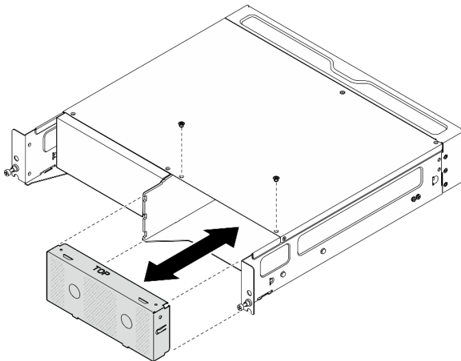
Figure 23. Installation de l'obturateur de nœud
