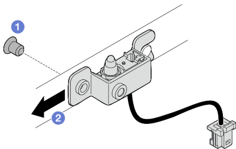
Figure 149. Retrait du commutateur d'intrusion avec câble
