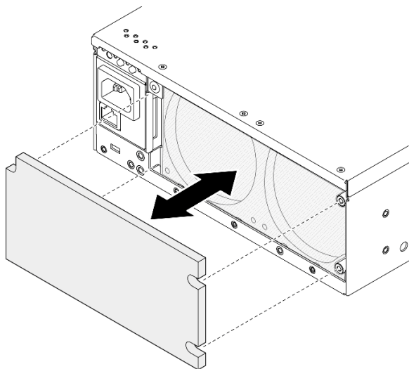
Figure 73. Retrait du filtre anti-poussière
