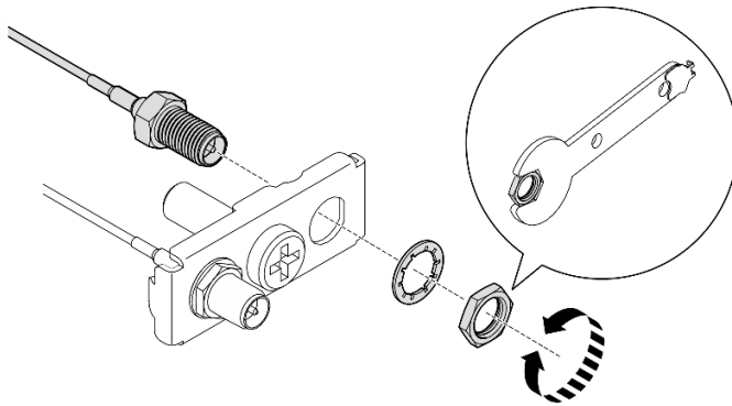
Figure 319. Desserrage des câbles du support
