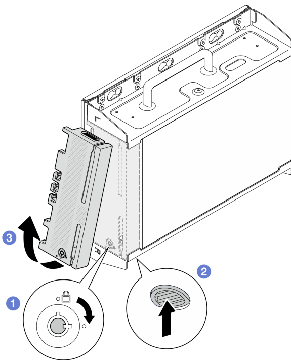
Figure 26. Retrait du panneau de sécurité
