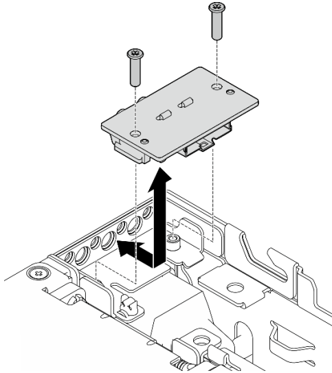
Figure 221. Installation du panneau opérateur arrière
