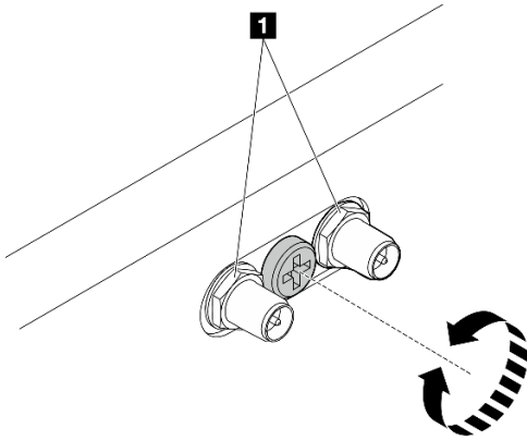
Figure 39. Raccourcissement des connecteurs SMA
