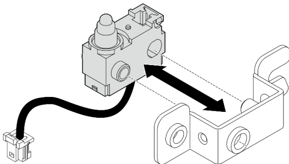
Figure 145. Insertion du commutateur d'intrusion dans le support
