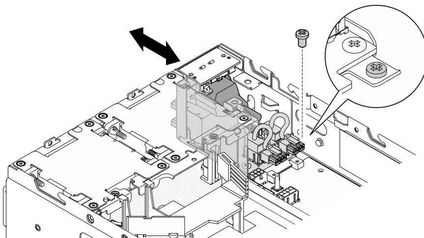
Figure 204. Installation du module PIB
