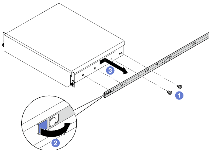
Figure 9. Retrait de la glissière interne
