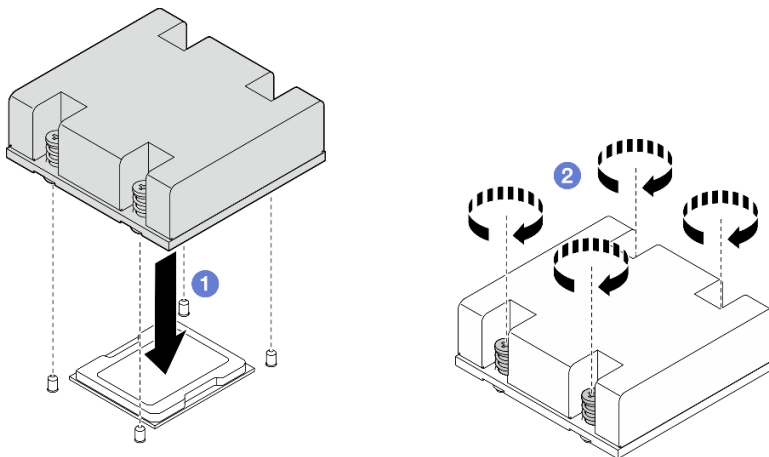
Figure 219. Installation du dissipateur thermique de processeur
