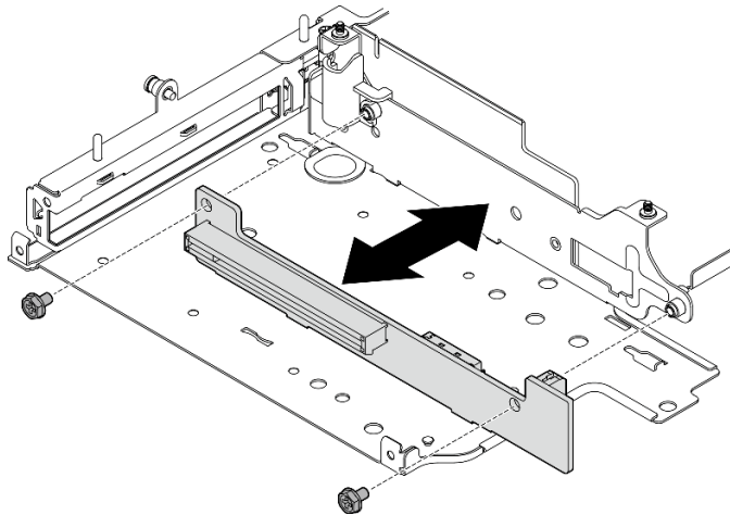
Figure 235. Retrait de la carte mezzanine
