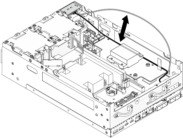
Figure 216. Placer le câble de signal
