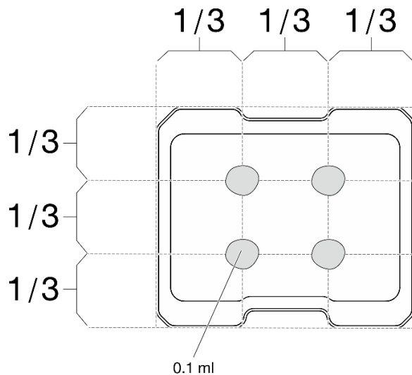
Figure 218. Forme correcte de la pâte thermoconductrice
