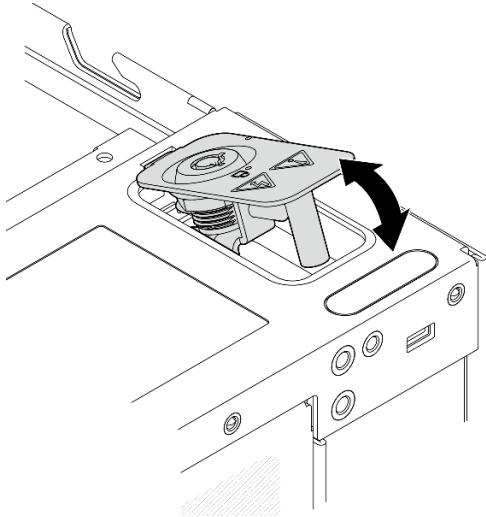
Figure 171. Installation du verrou de sécurité du système
