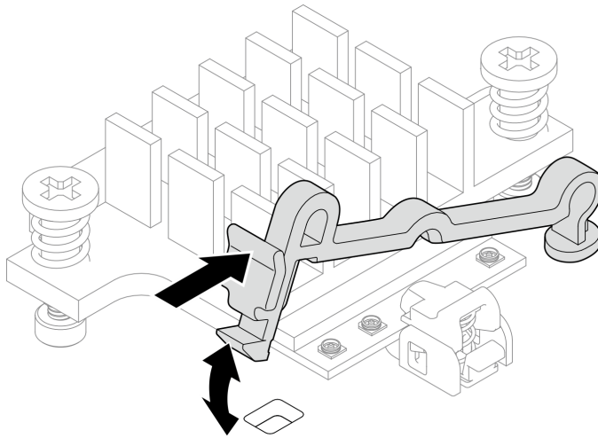
Figure 328. Soulever le support de câble
