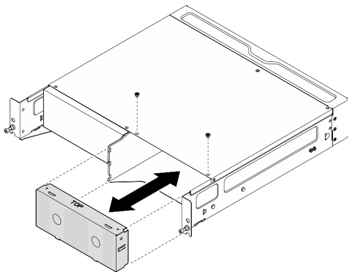
Figure 5. Installation de l'obturateur de nœud
