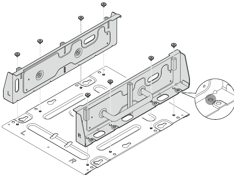
Figure 59. Démontez le support du nœud
