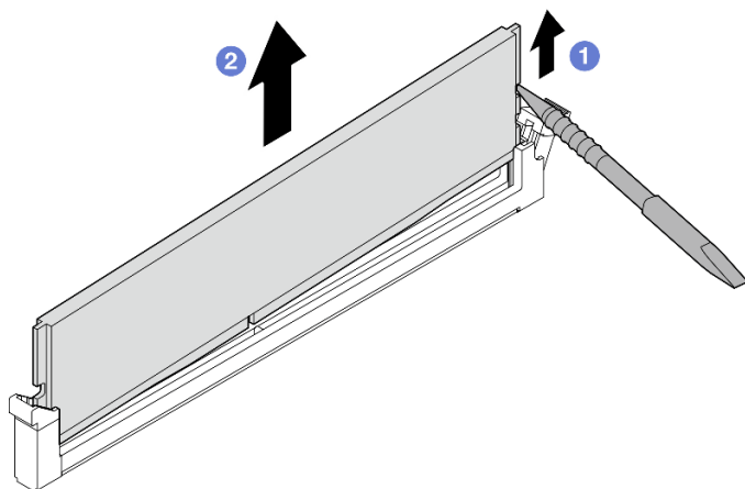
Figure 178. Retrait du module de mémoire
