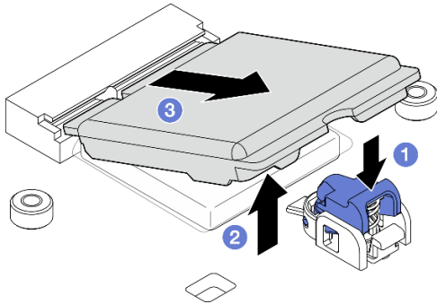
Figure 285. Retrait du carter factice
