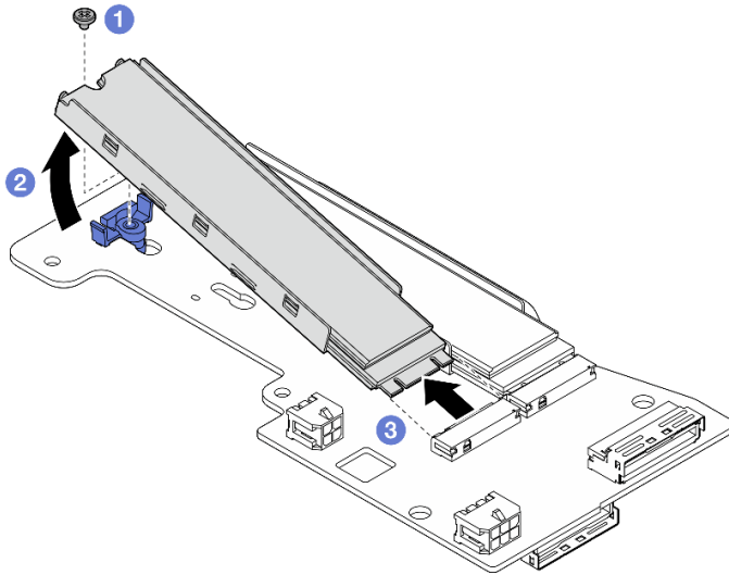
Figure 226. Retrait d'une unité M.2
