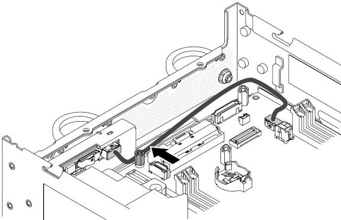
Figure 341. Cheminement des câbles du panneau opérateur avant
