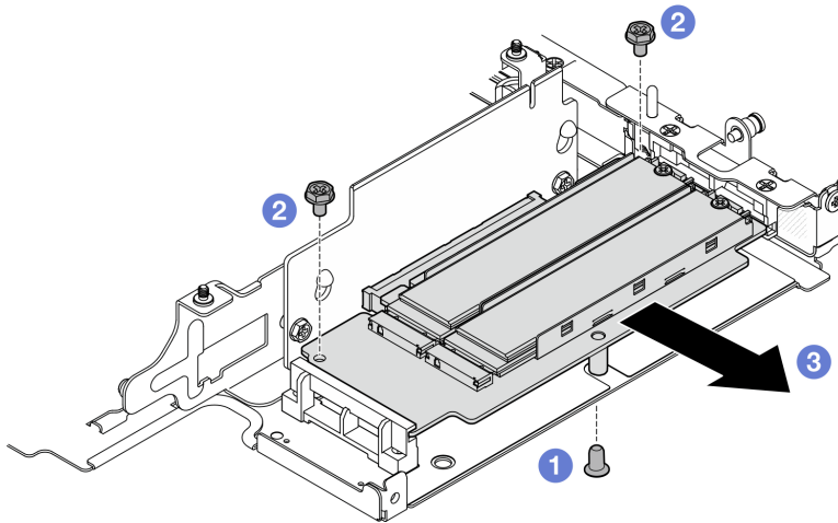
Figure 236. Retrait de l'adaptateur M.2
