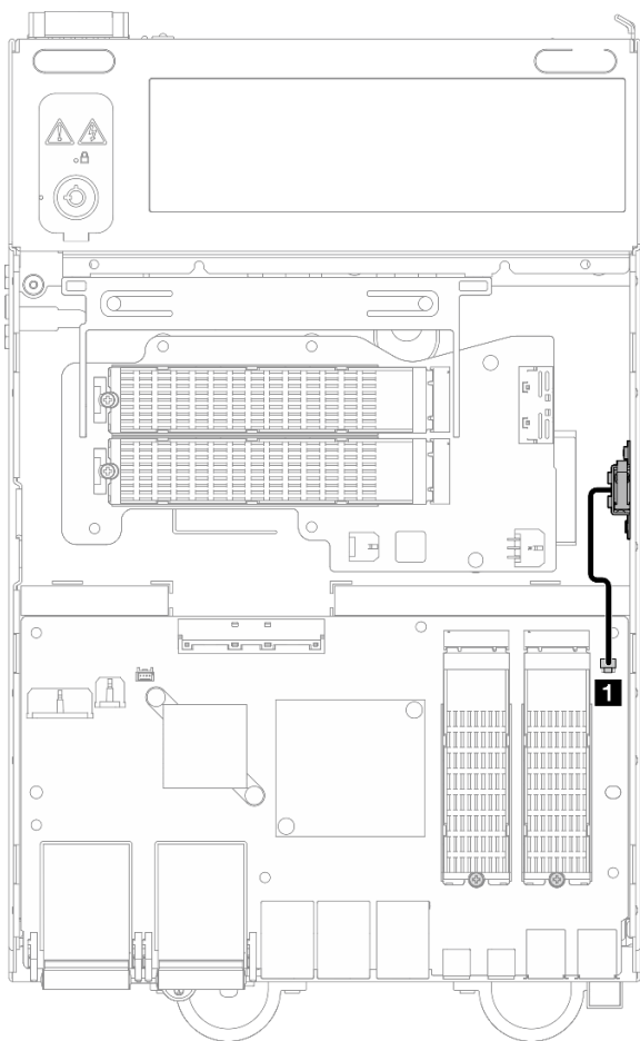
Figure 148. Cheminement des câbles du commutateur d'intrusion inférieure
