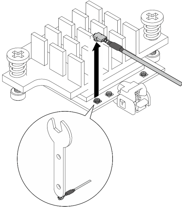
Figure 96. Déconnexion du câble
