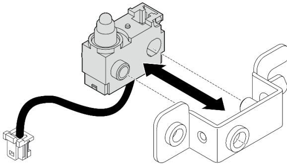
Figure 151. Insertion du commutateur d'intrusion dans le support
