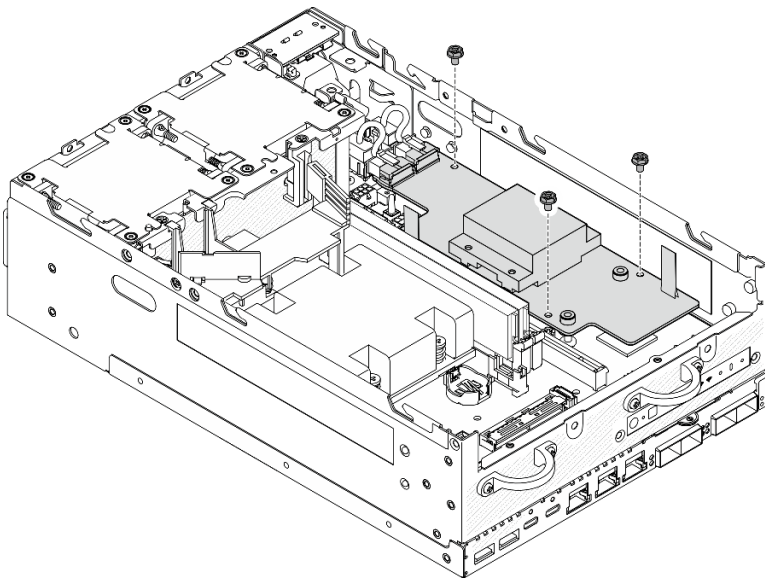
Figure 209. Desserer les vis
