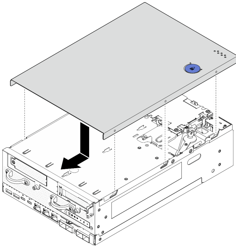
Figure 188. Installation du carter supérieur
