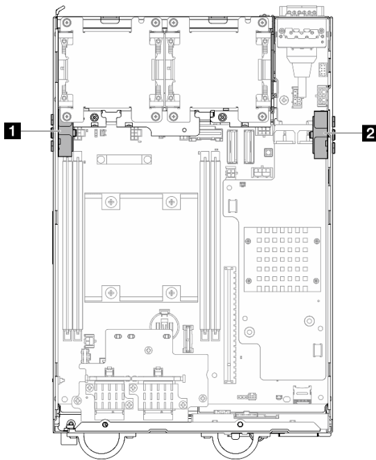
Figure 323. Lieux d'assemblages SMA
