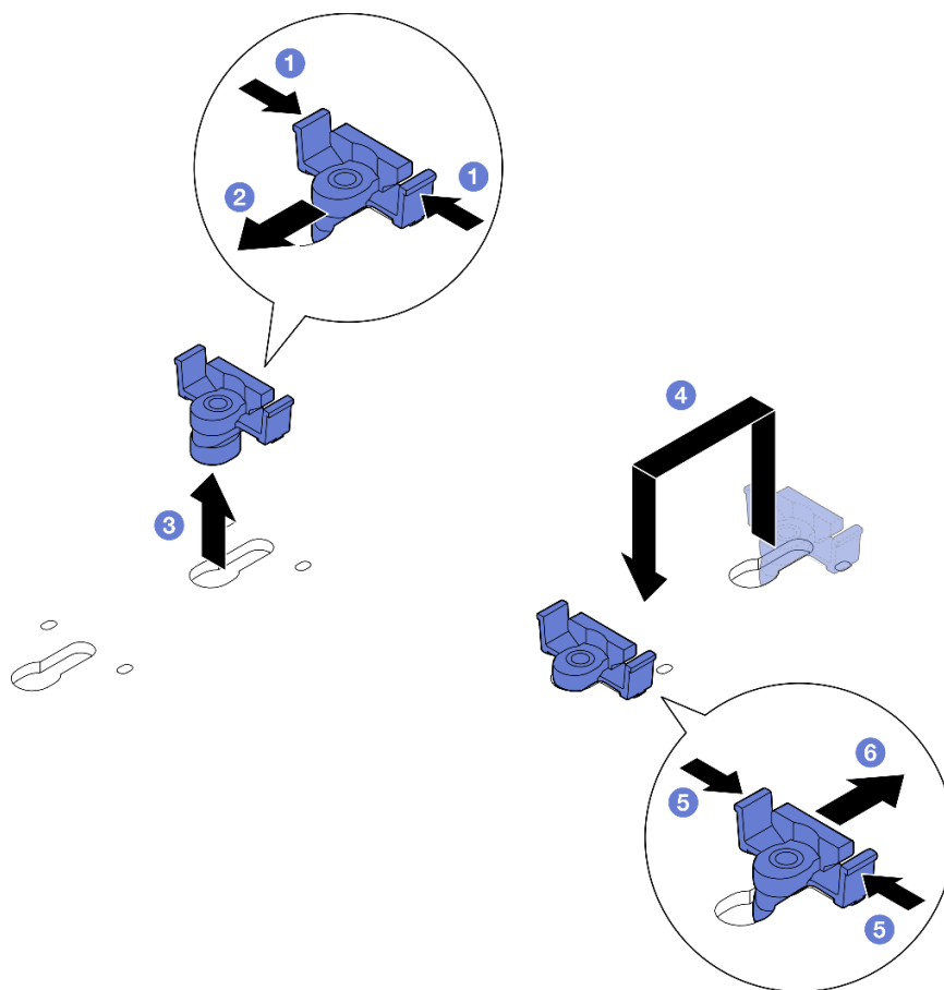
Figure 114. Ajustez le crochet de retenue M.2
