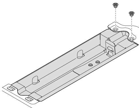
Figure 258. Installation du boîtier du module de géolocalisation
