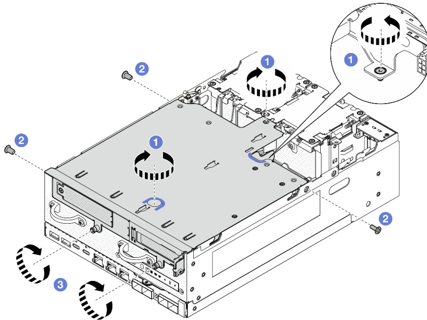
Figure 265. Fixer l'assemblage de carte mezzanine
