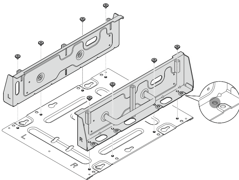
Figure 34. Assemblage du manchon de nœud
