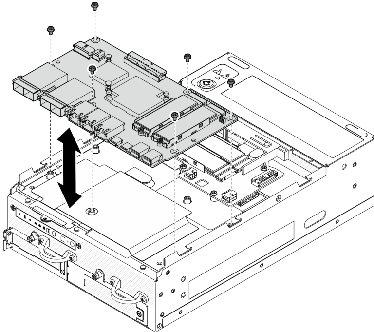
Figure 160. Installation de la carte de module d'E/S
