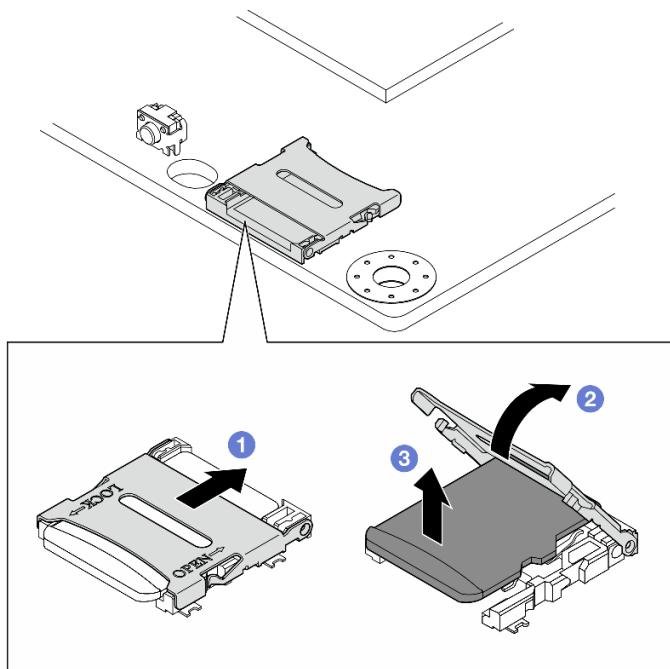
Figure 182. Retrait de la carte microSD
