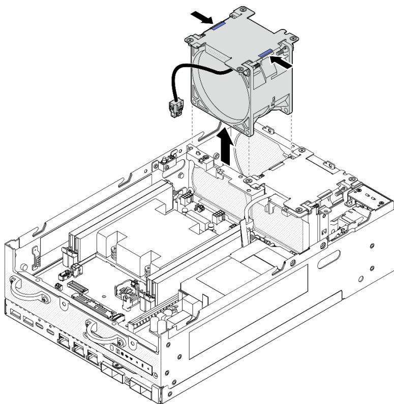
Figure 127. Retrait du module de ventilation
