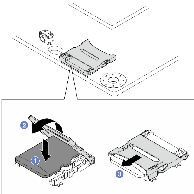
Figure 183. Installation de la carte MicroSD
