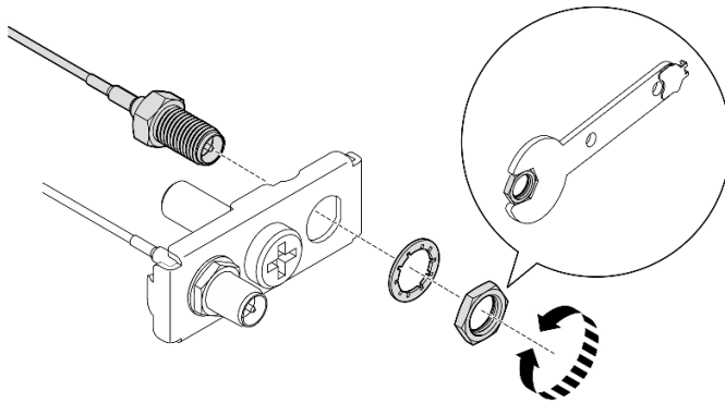
Figure 308. Desserrage des câbles du support
