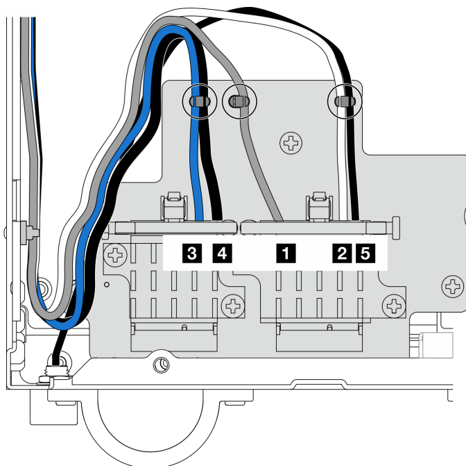
Figure 343. Cheminement des câbles de l'antenne WLAN et de l'antenne Bluetooth
