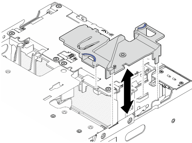
Figure 85. Installation de la grille d'aération
