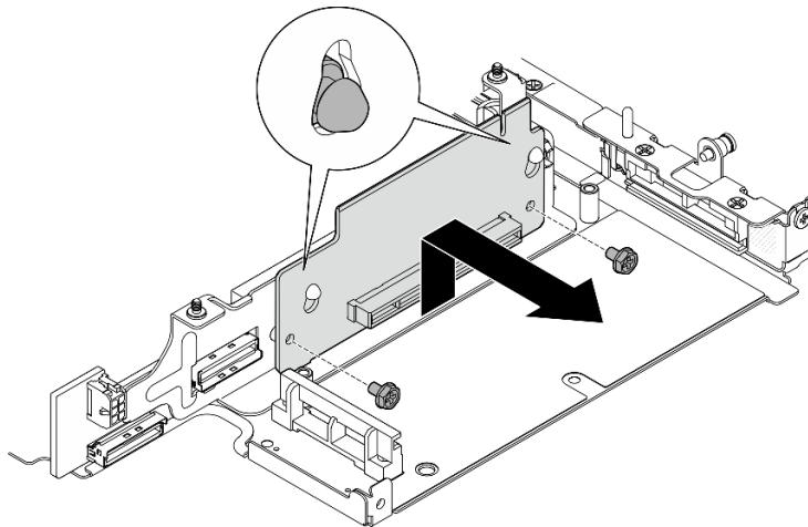
Figure 237. Retrait de la carte mezzanine
