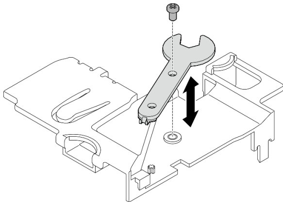
Figure 298. Désengagement de la clé
