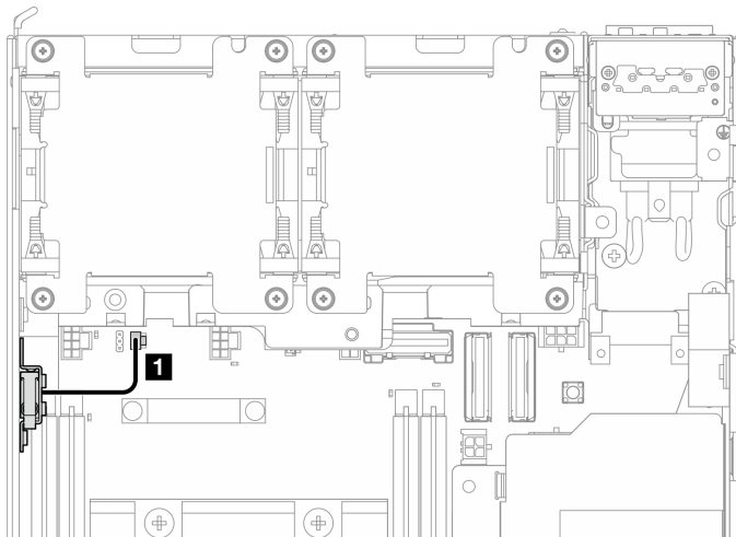
Figure 147. Cheminement des câbles du commutateur d'intrusion supérieur
