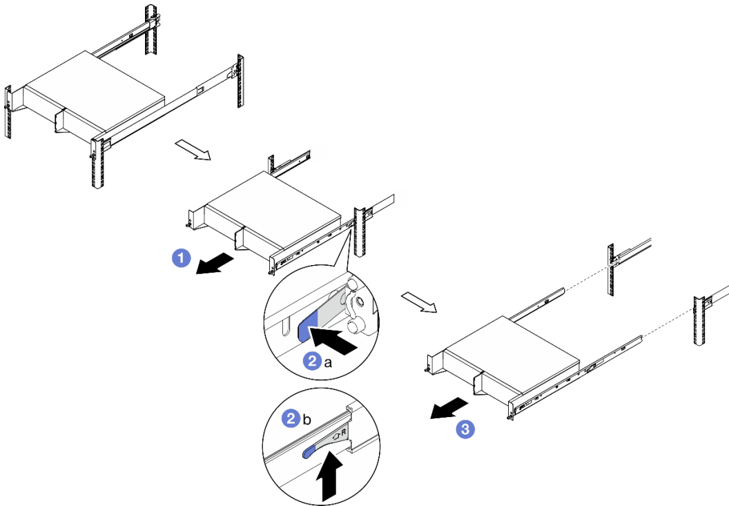
Figure 8. Retrait du boîtier de l'armoire
