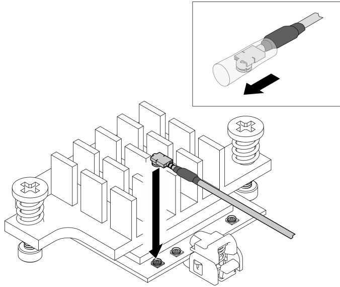
Figure 331. Connexion du câble
