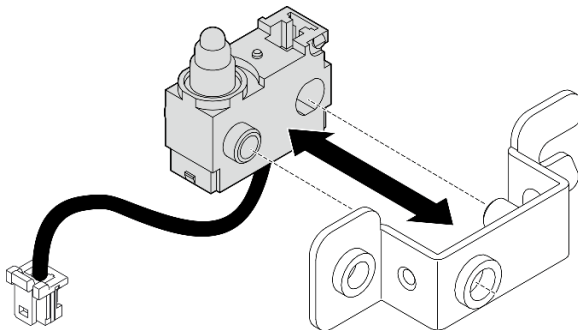
Figure 144. Séparation du commutateur d'intrusion du support
