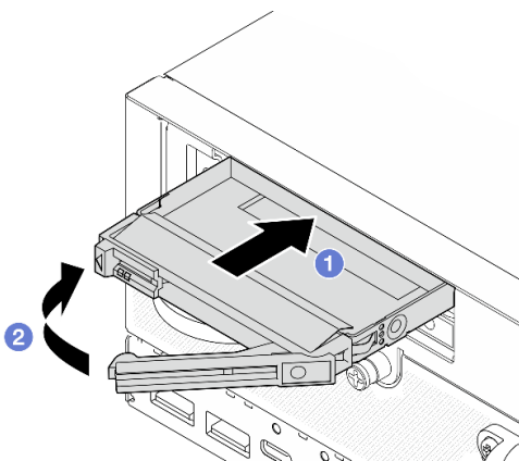
Figure 80. Installation d'un obturateur d'unité
