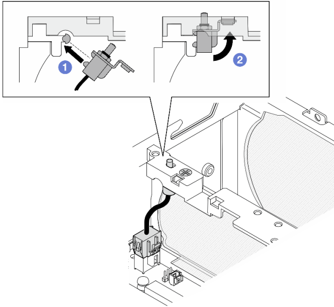
Figure 124. Installation du commutateur d'intrusion avec câble
