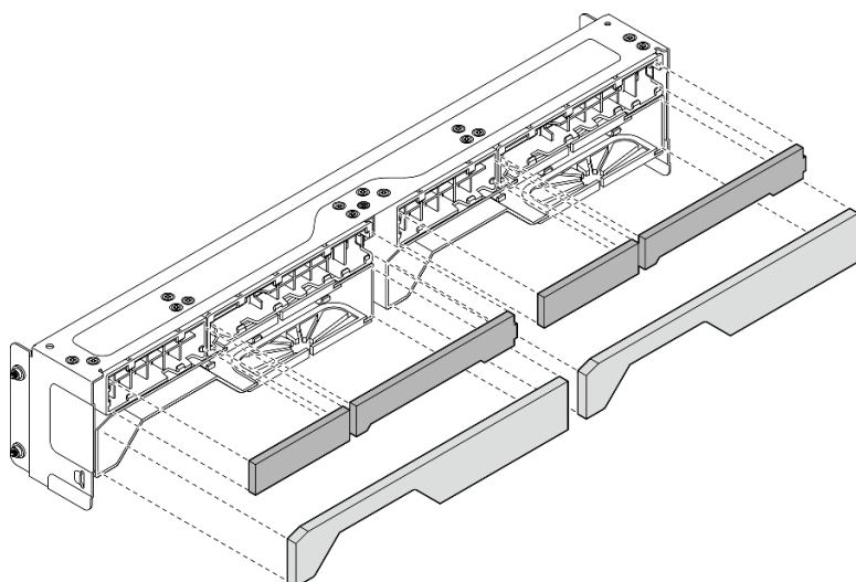
Figure 68. Retrait des filtres anti-poussière
