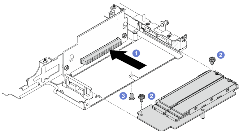
Figure 243. Installation de l'adaptateur M.2
