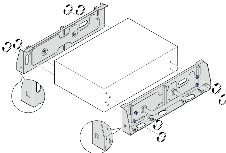
Figure 33. Desserrage des vis serrage à main pour retirer les supports latéraux
