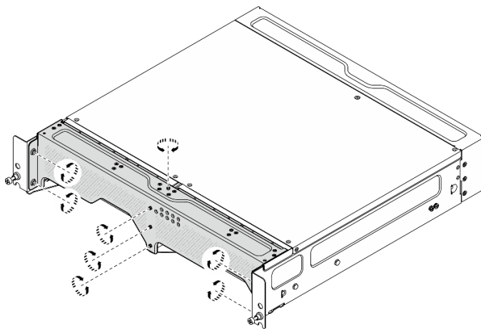
Figure 25. Serrer les vis
