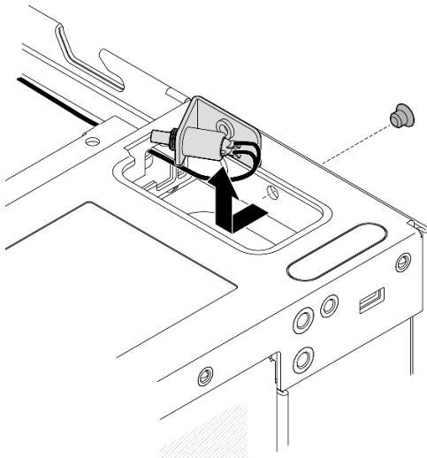
Figure 168. Retrait du commutateur en position verrouillée avec câble
