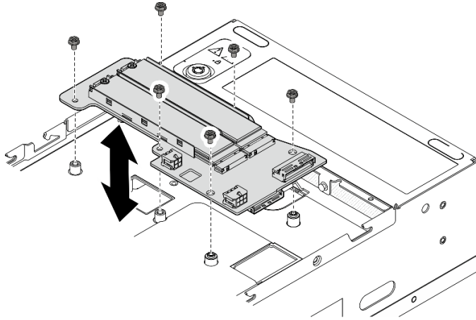
Figure 113. Retrait de l'adaptateur câblé M.2 inférieur
