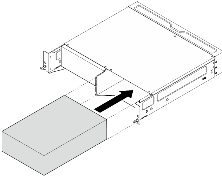
Figure 22. Installation du nœud
