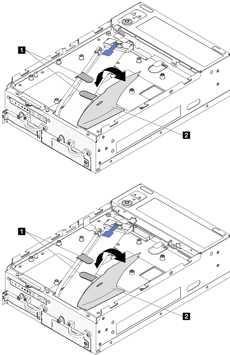
Figure 159. Cheminement des câbles de la carte d'E/S
