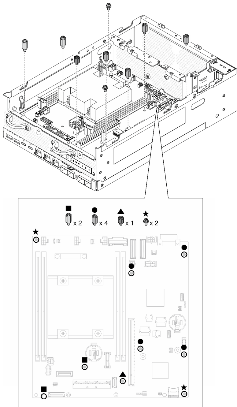
Figure 272. Les vis et les supports de la carte mère
