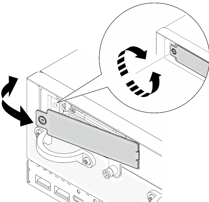
Figure 81. Installation du panneau
