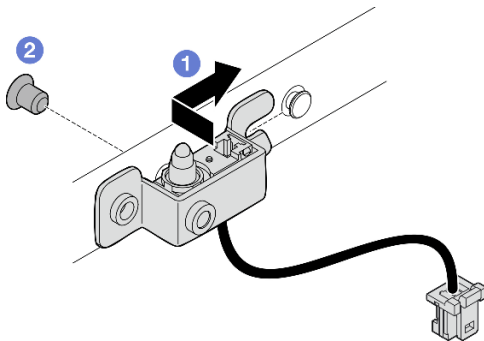
Figure 152. Installation du commutateur d'intrusion avec câble
