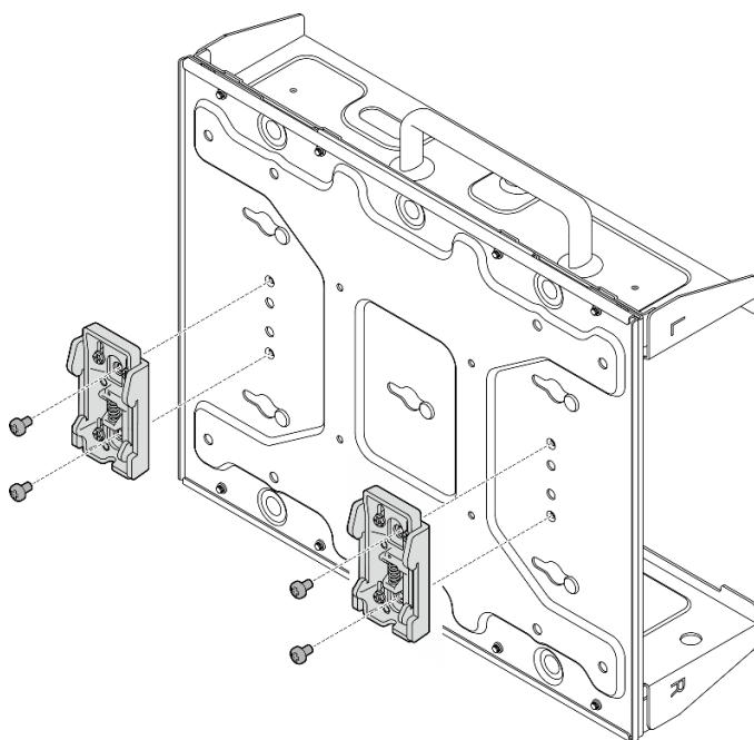
Figure 53. Retrait des clips de la glissière DIN
