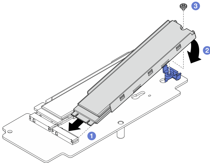
Figure 241. Installation d'une unité M.2
