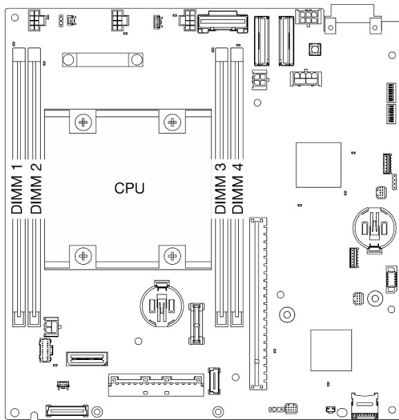
Figure 1. Disposition des modules de mémoire et des processeurs
