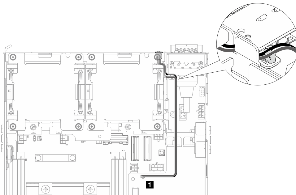
Figure 200. Câble du voyant d'état du PMB se connectant à la carte du module d'alimentation CC (PMB CC)
