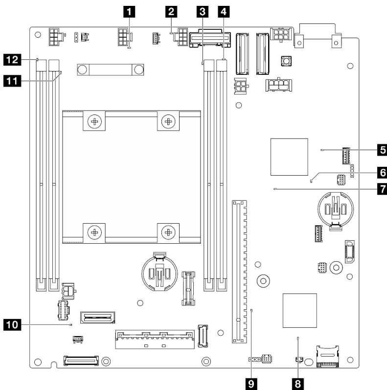
Figure 351. Voyants de la carte mère
