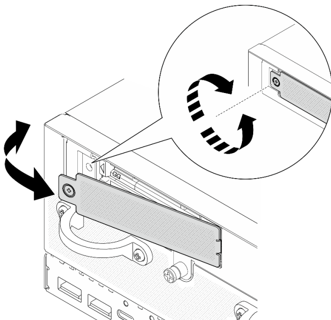
Figure 76. Retrait du panneau
