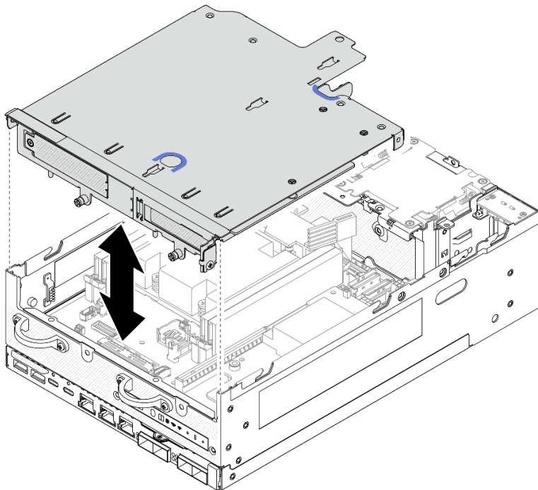
Figure 266. Abaisser l'assemblage de carte mezzanine
