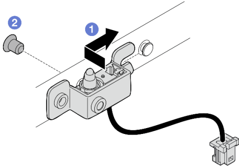
Figure 146. Installation du commutateur d'intrusion avec câble
