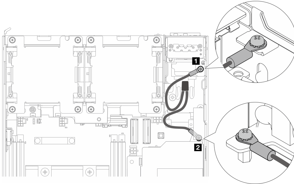
Figure 140. Connexion du câble de mise à la terre
