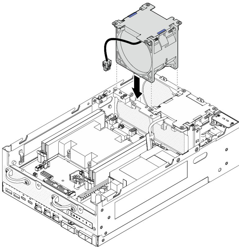
Figure 128. Installation du module de ventilation
