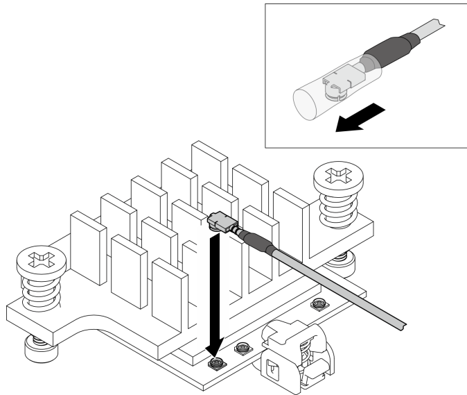
Figure 291. Connexion du câble
