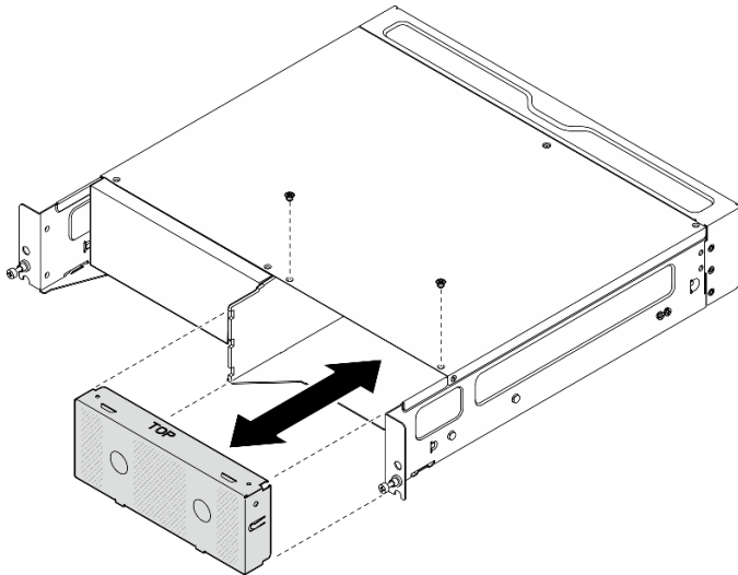
Figure 21. Retrait de l'obturateur de nœud
