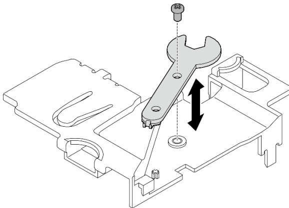
Figure 92. Désengagement de la clé
