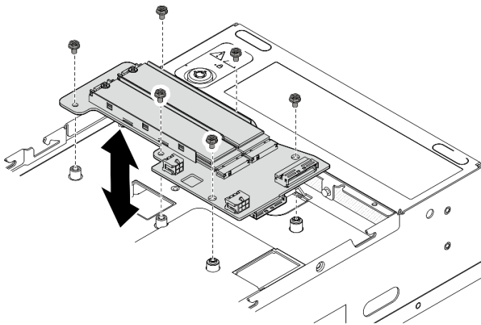
Figure 115. Installation de l'adaptateur câblé M.2 inférieur
