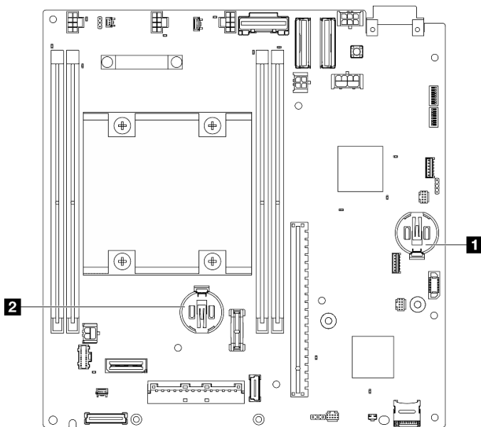
Figure 120. Emplacements de la pile CMOS sur la carte mère
