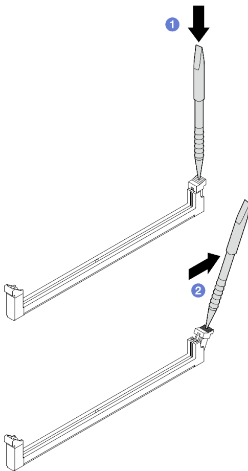
Figure 177. Ouverture d'une patte de retenue
