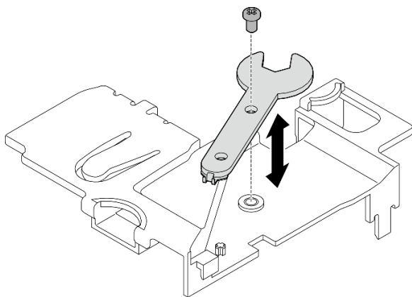
Figure 101. Rangement de la clé
