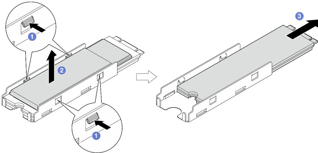
Figure 173. Retrait du dissipateur thermique M.2
