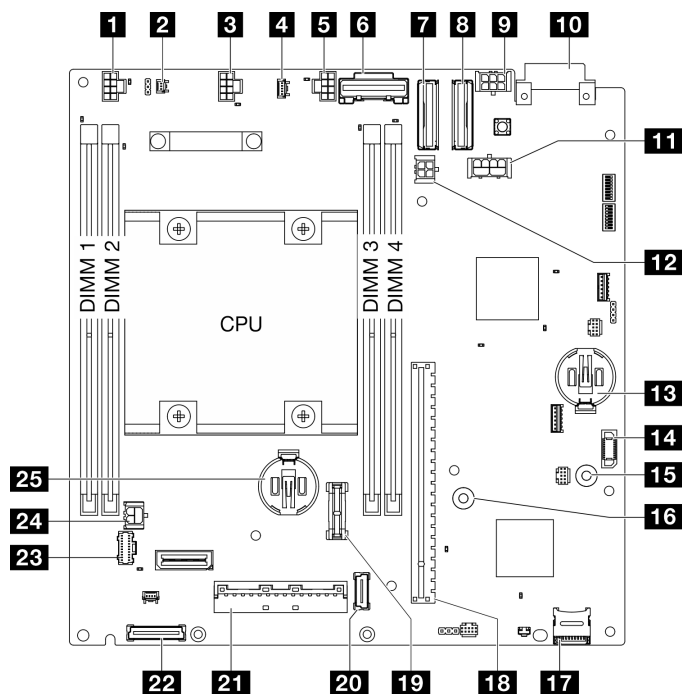
Figure 346. Connecteurs de la carte mère
