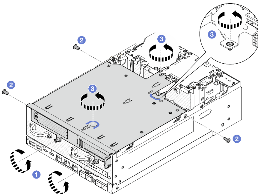
Figure 222. Retrait de l'assemblage de carte mezzanine
