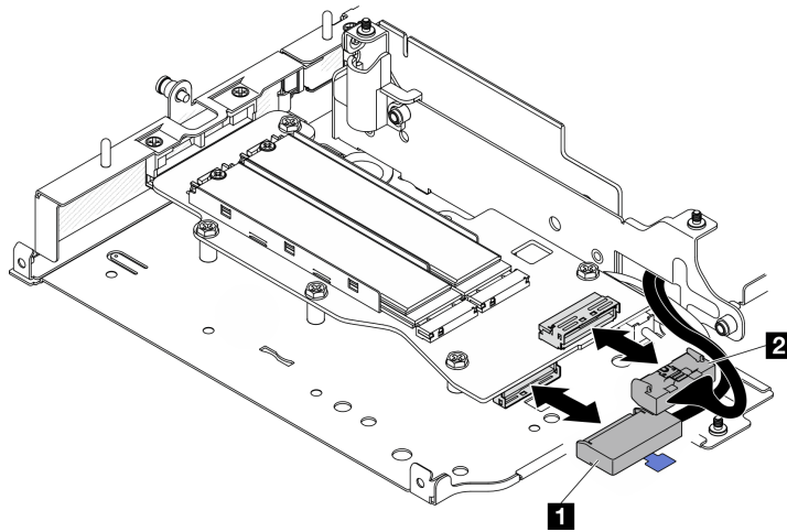
Figure 249. Débranchement du câble de signal
