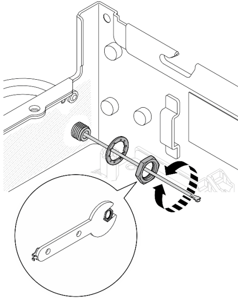
Figure 99. Retrait de l'antenne Bluetooth
