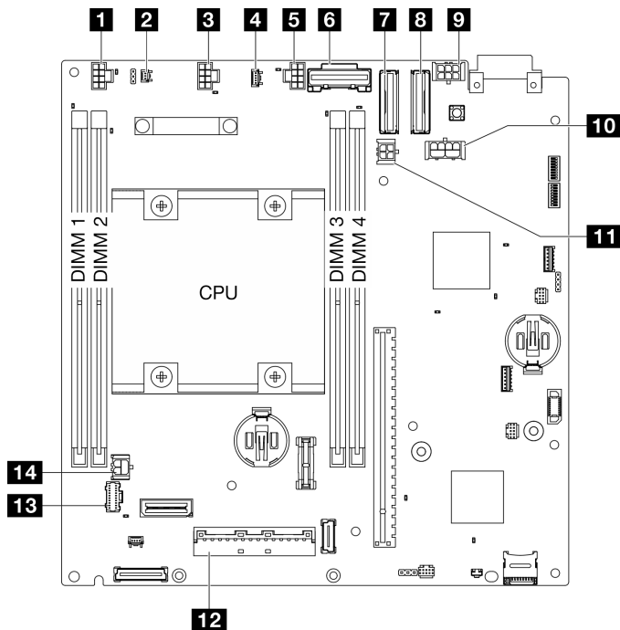
Figure 340. Connecteurs de la carte mère
