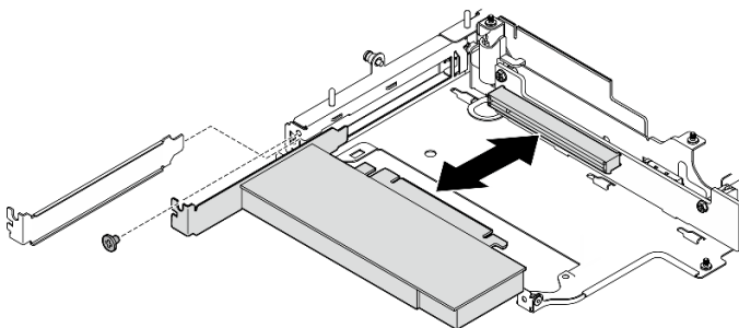
Figure 255. Installation de l'adaptateur PCIe
