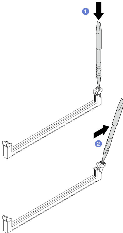
Figure 180. Ouverture d'une patte de retenue
