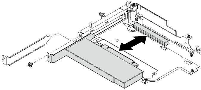
Figure 234. Retrait de l'adaptateur PCIe
