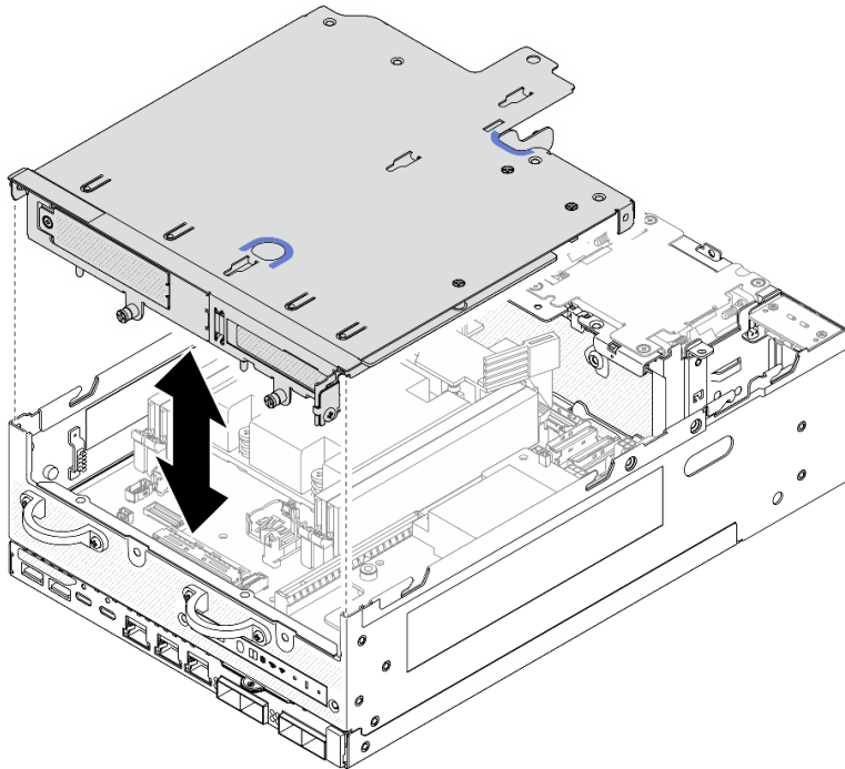
Figure 260. Abaisser l'assemblage de carte mezzanine
