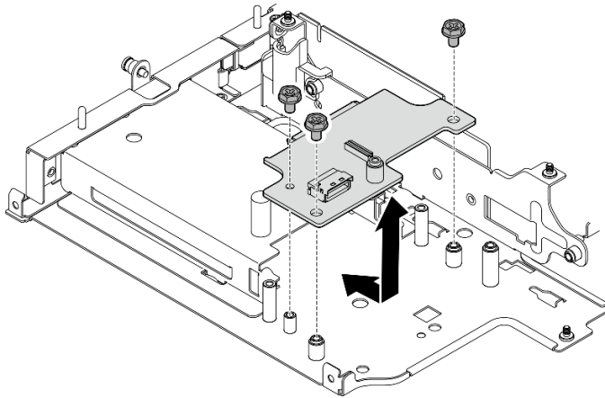
Figure 230. Retrait du fond de panier 1
