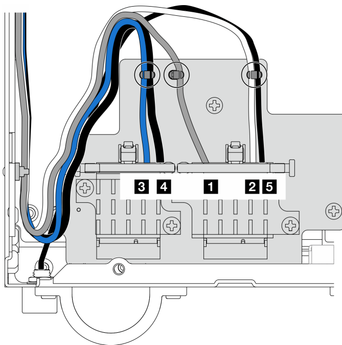
Figure 334. Cheminement des câbles pour l'adaptateur sans fil
