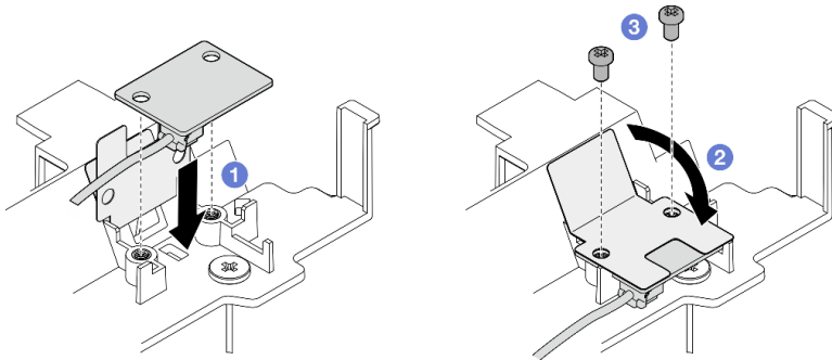
Figure 90. Installation de la carte du capteur de ventilation
