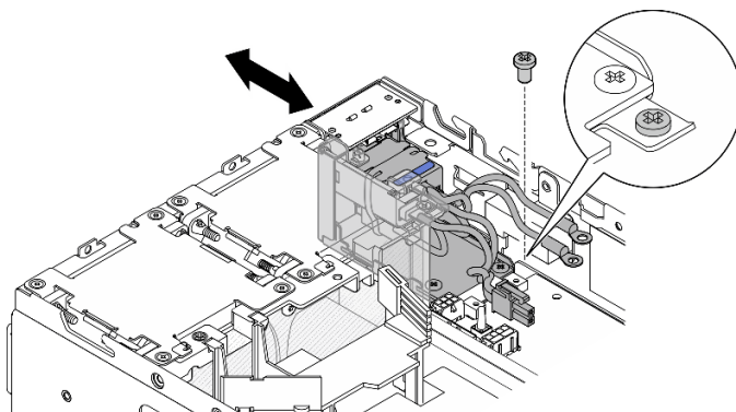
Figure 203. Retrait du module PIB CA
