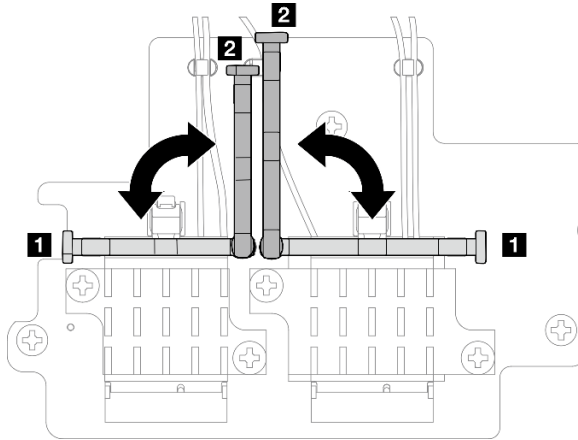
Figure 313. Faire pivoter le support de câble
