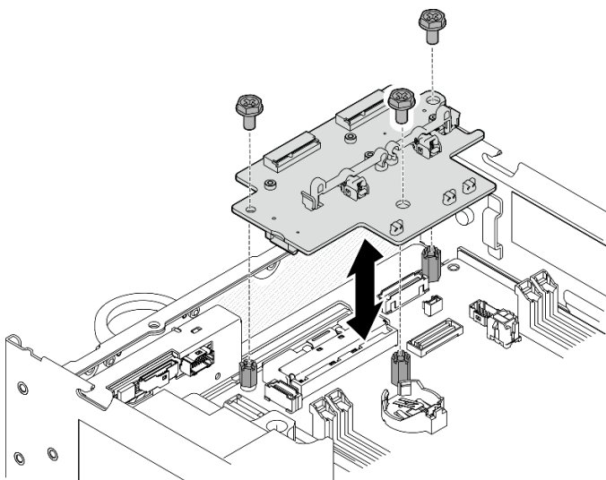
Figure 110. Installation de l'adaptateur sans fil
