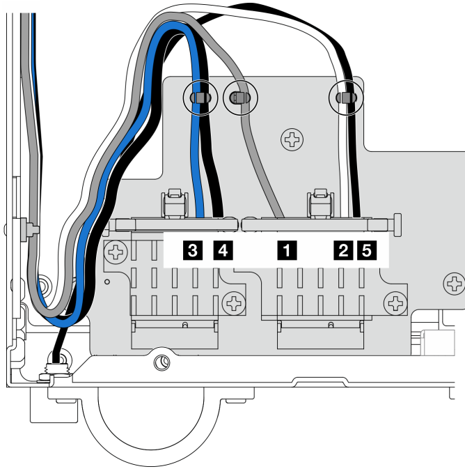
Figure 290. Cheminement des câbles pour l'adaptateur sans fil
