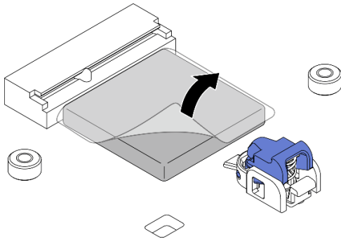
Figure 286. Retrait du film du tampon thermique
