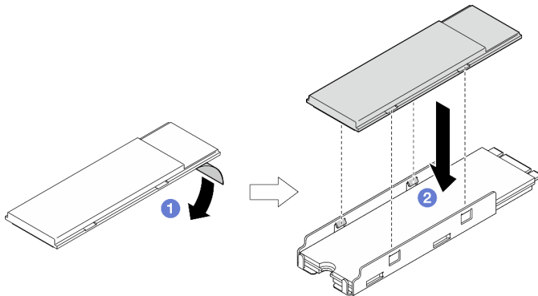
Figure 175. Installation du dissipateur thermique M.2
