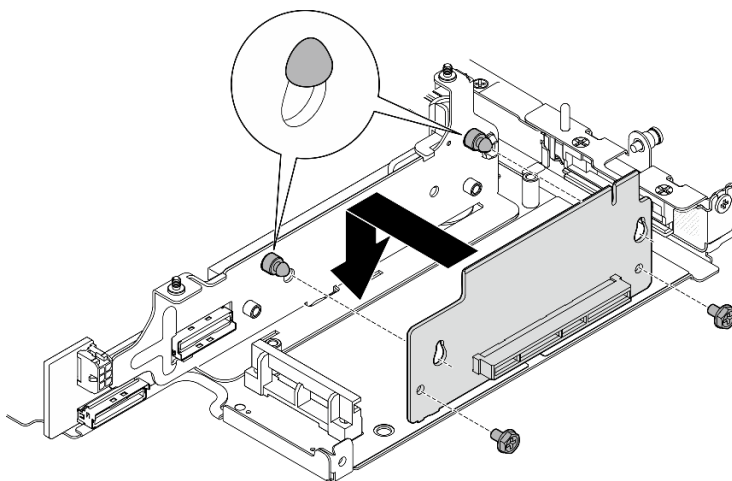
Figure 242. Installation de la carte mezzanine
