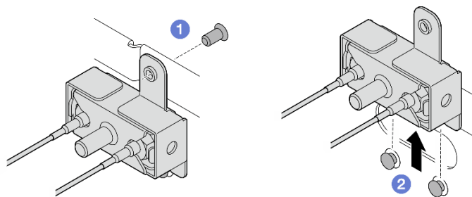
Figure 306. Retrait de l'assemblage SMA
