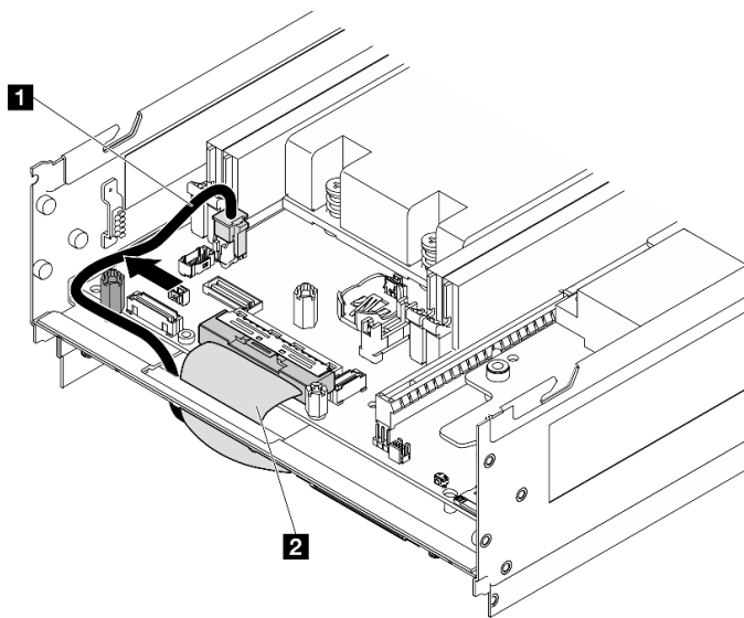
Figure 157. Cheminement des câbles de la carte d'E/S
