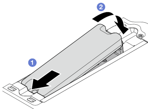
Figure 259. Installation du module de géolocalisation
