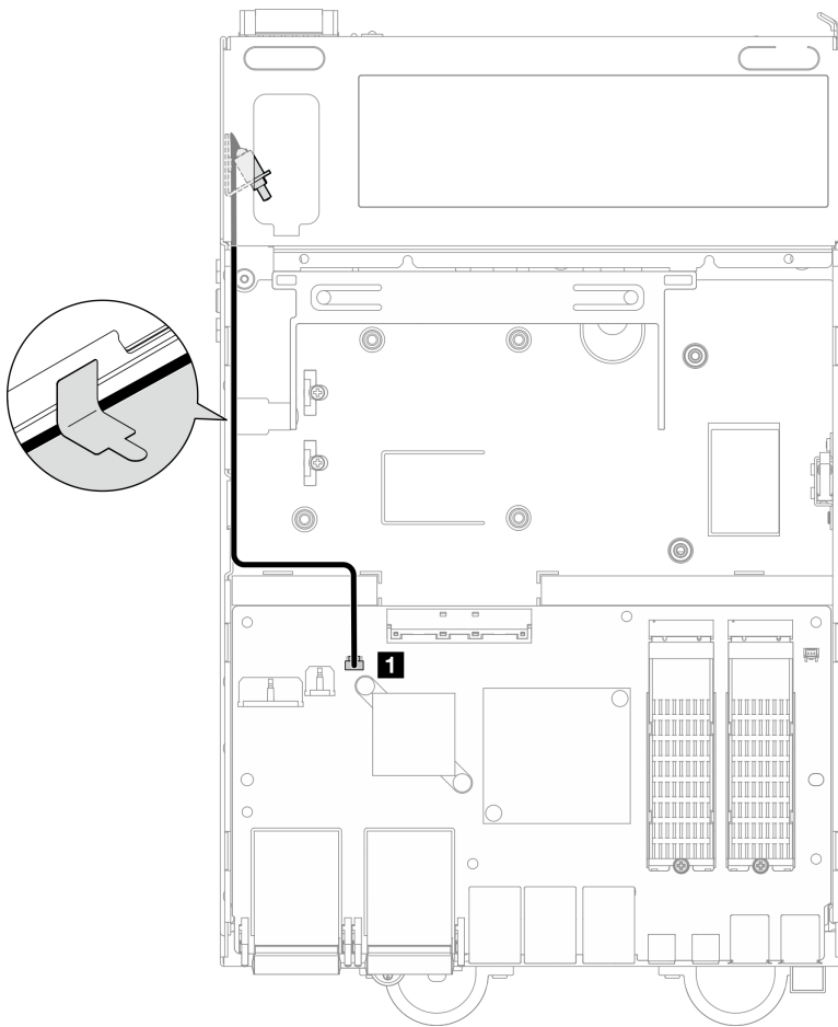
Figure 167. Cheminement des câbles du commutateur en position verrouillée
