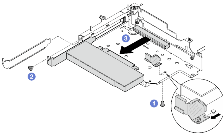
Figure 227. Retrait de l'adaptateur PCIe
