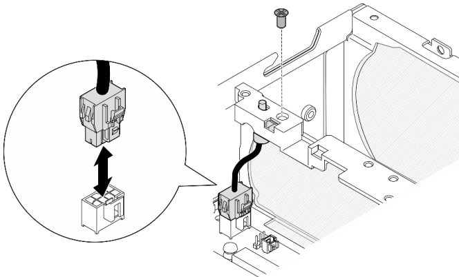
Figure 125. Installation du commutateur de direction du ventilateur
