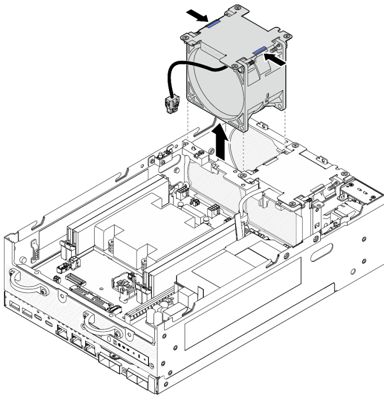
図127. ファン・モジュールの取り外し
