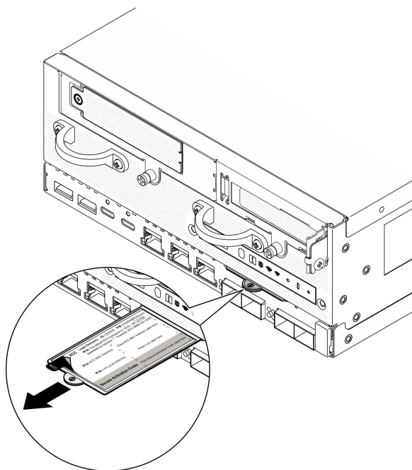
図 277. 引き出し式情報タブにある Lenovo XClarity Controller のネットワーク・アクセス・ラベル
