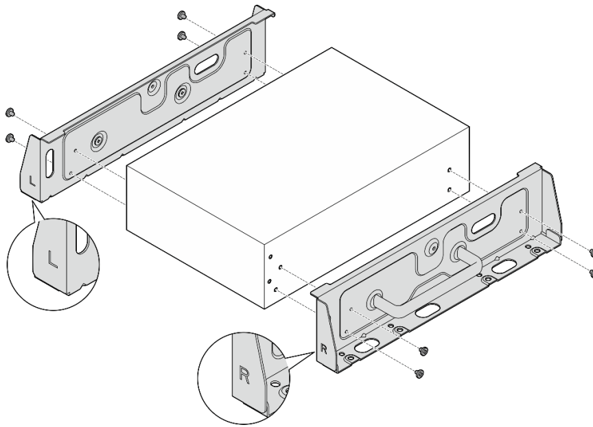
図40. ねじでのサイド・ブラケットの取り付け
