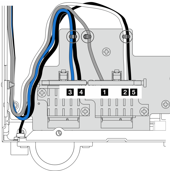
図 343. WLAN アンテナおよび Bluetooth アンテナのケーブル配線
