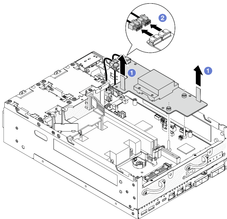
図 210. 電源モジュール・ボードの取り外し
