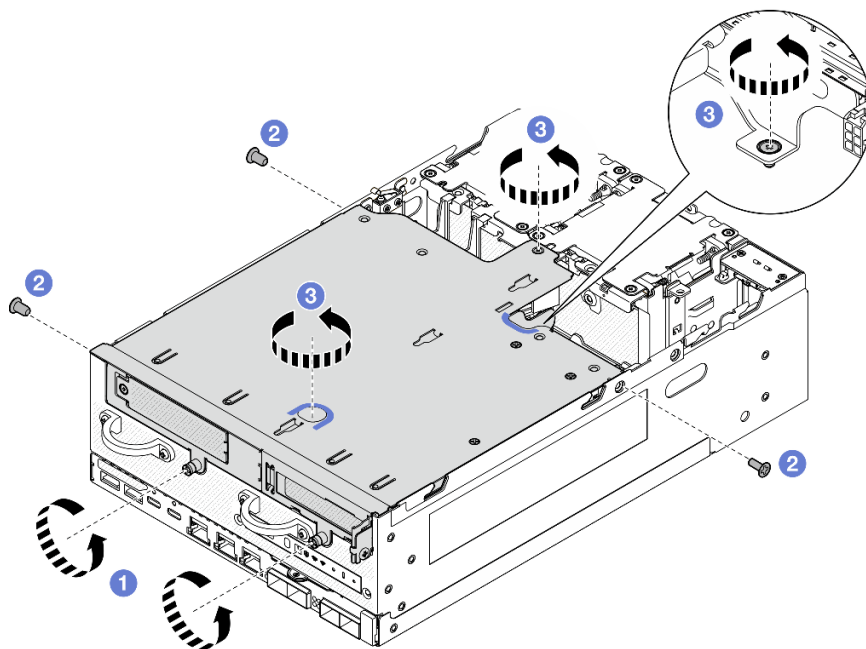
図 222. ライザー・アセンブリーの取り外し
