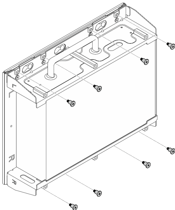
図 48. ノード・ブラケットの取り付け
