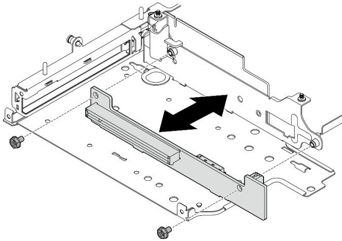
図 250. ライザー・カードの取り付け
