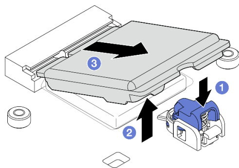
図 285. ダミー・カバーの取り外し
