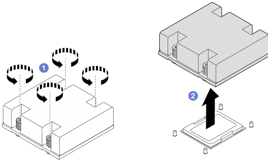
図217. プロセッサ・ヒートシンクの取り外し
