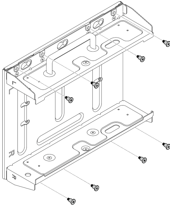
図27. ノード・ブラケットの取り外し
