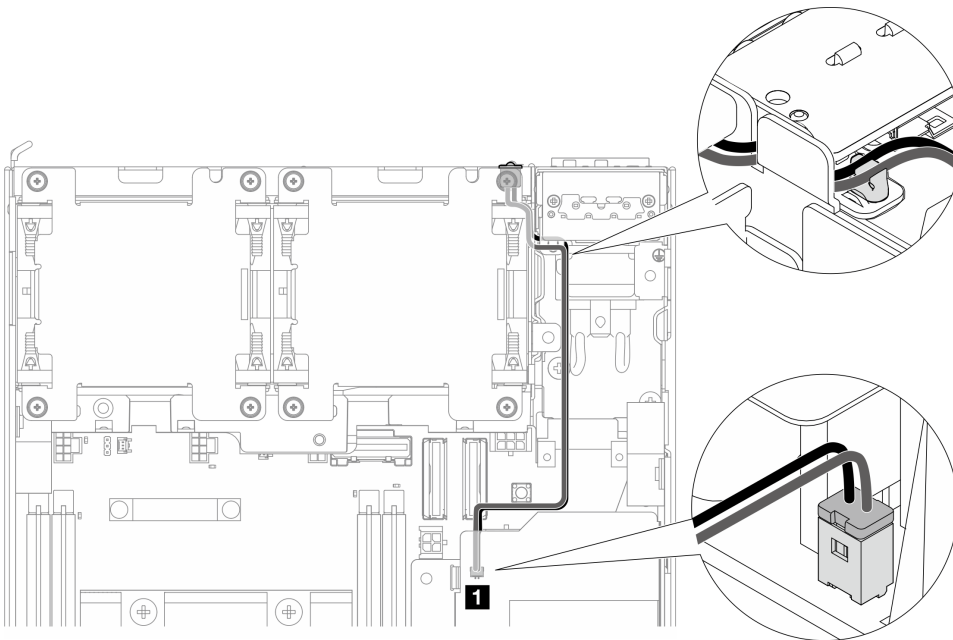
図 201. 内部パワー・サプライ・ユニット (AC PMB) に接続する PMB 状況 LED ケーブル
