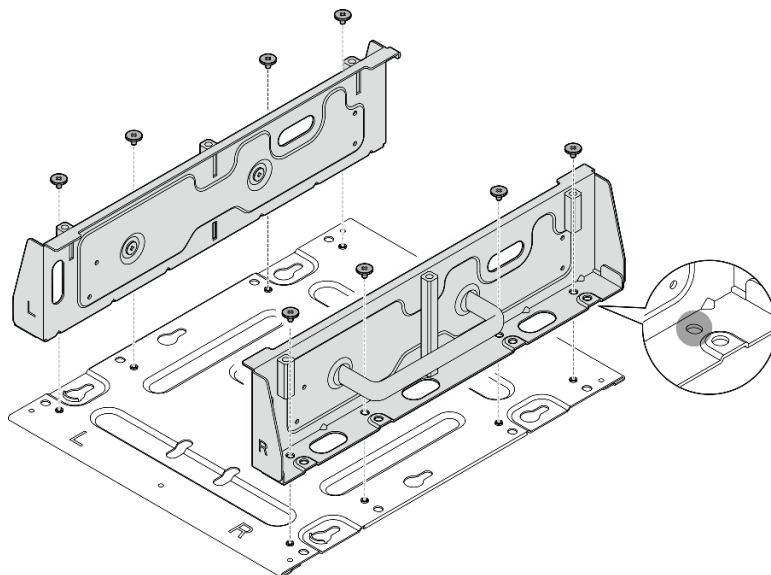
図 59. ノード・ブラケットの分解
