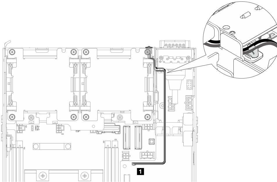
図 200. DC 電源モジュール・ボード (DC PMB) に接続する PMB 状況 LED ケーブル
