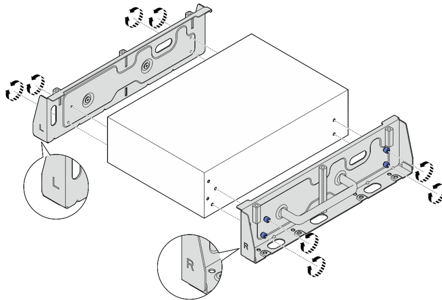
図41. つまみねじでのサイド・ブラケットの取り付け
