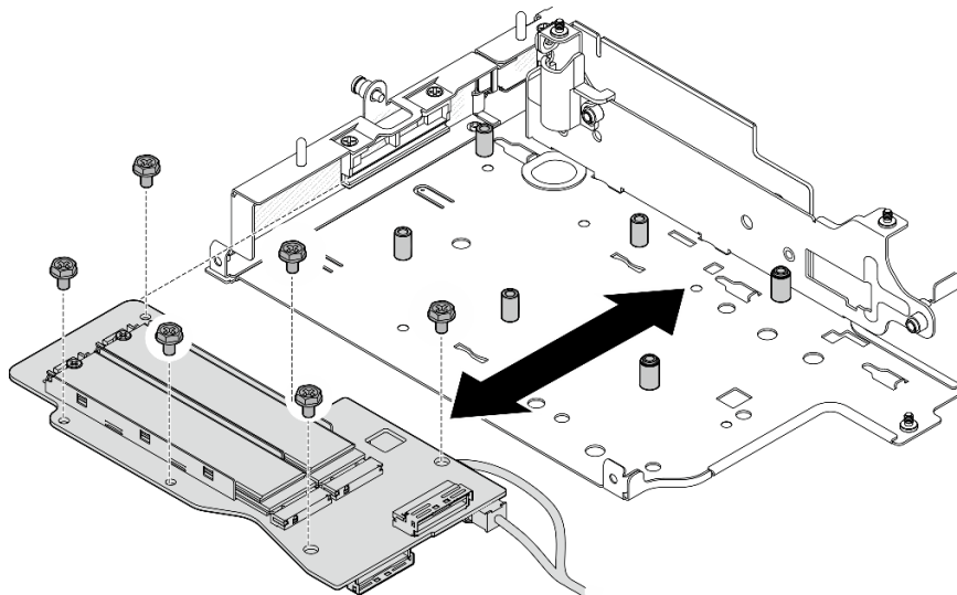
図 225. M.2 ケーブル接続アダプターの取り外し
