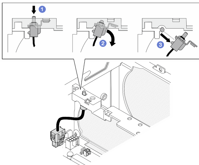
図 123. ファン方向スイッチの取り外し
