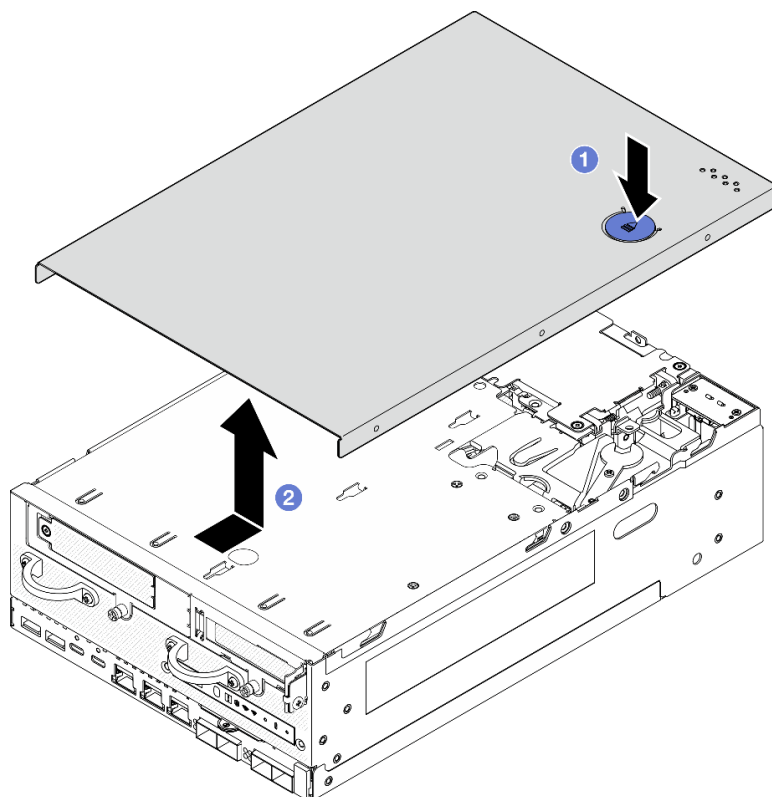
図185. トップ・カバーの取り外し
