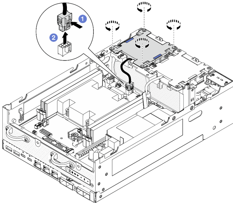
図126. ファン・モジュールの取り外し
