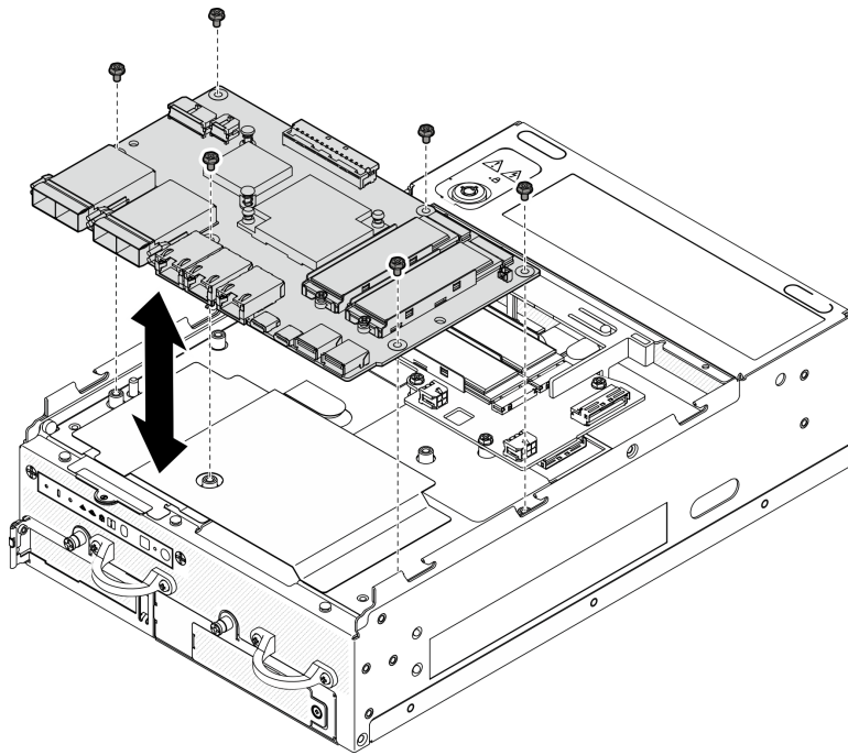
図155. I/O モジュール・ボードの取り外し
