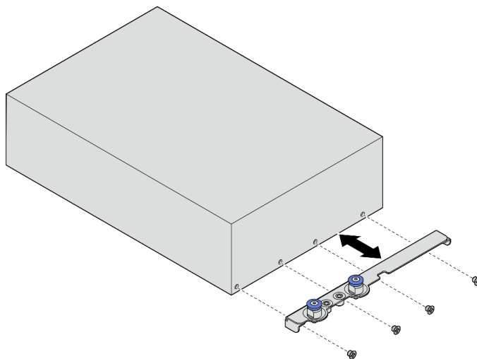
図6. エンクロージャー・ブラケットの取り外し
