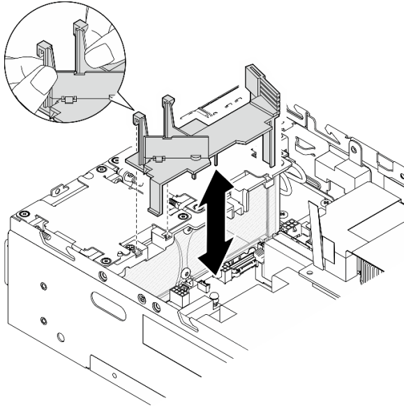
図 86. エアー・バッフルの取り外し
