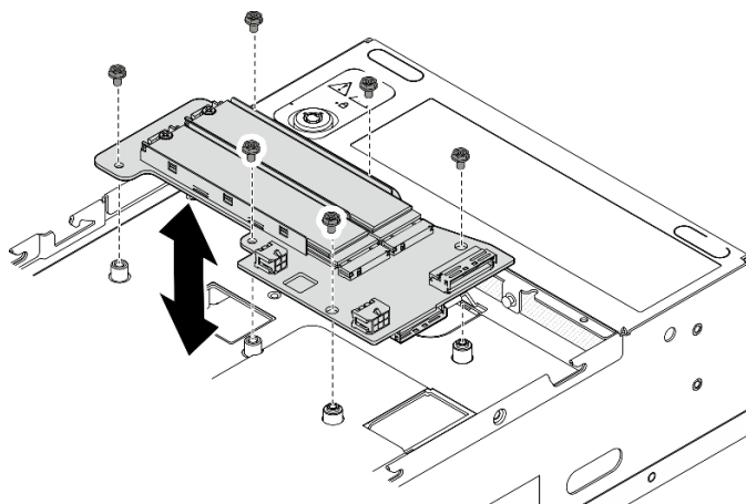
図 115. 下部の M.2 ケーブル接続アダプターの取り付け
