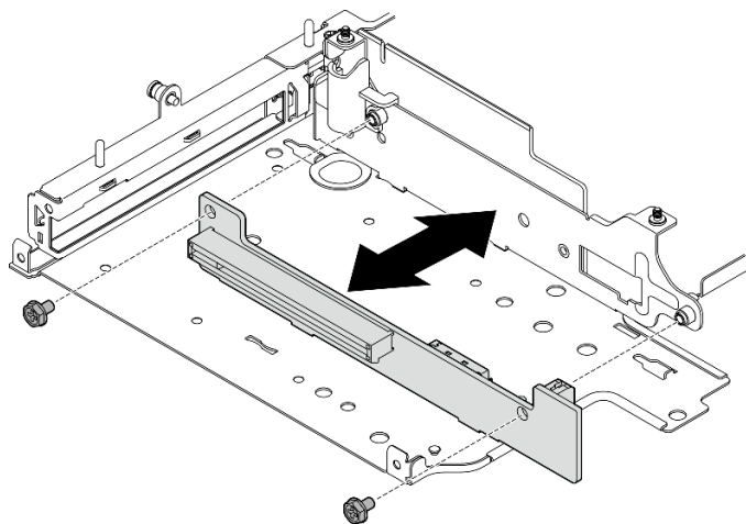
図235. ライザー・カードの取り外し
