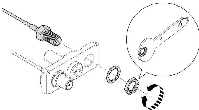
図 308. ブラケットからケーブルを緩める
