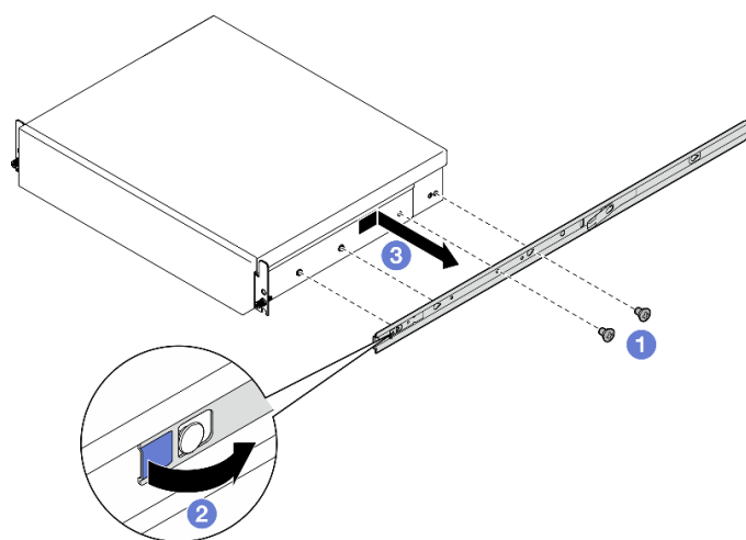
図9. 内側レールの取り外し
