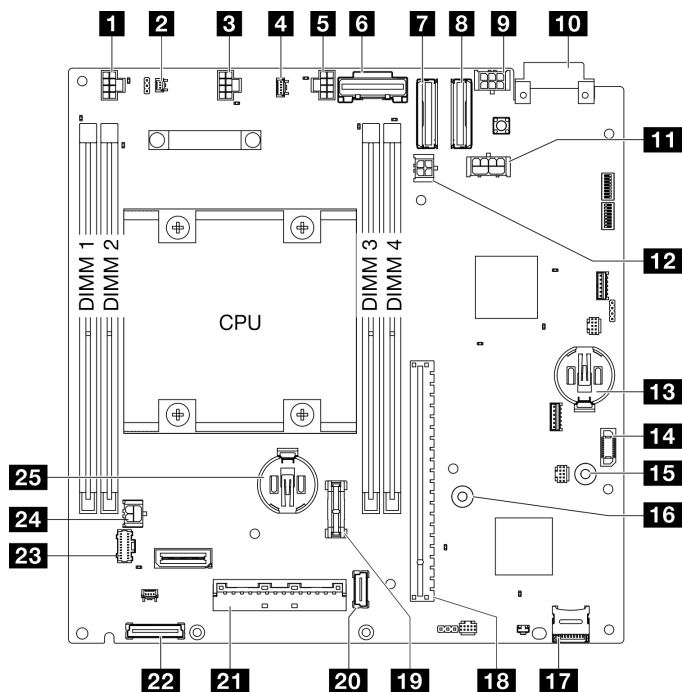
図 346. システム・ボード・コネクタ
