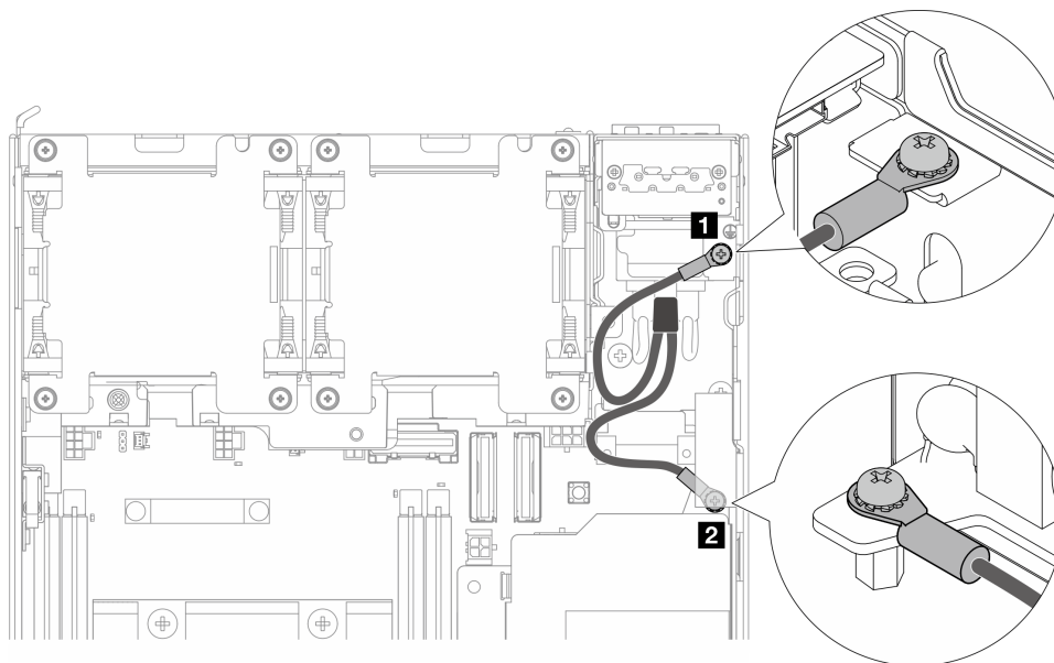
図 133. 接地用ケーブルの取り外し
