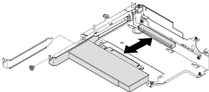
図234. PCIe アダプターの取り外し
