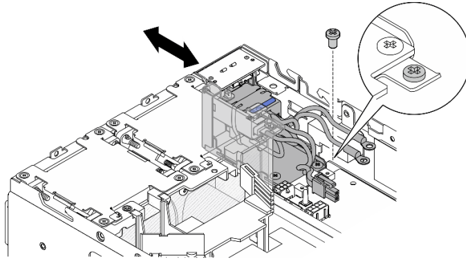
図206. PIB モジュールの取り付け
