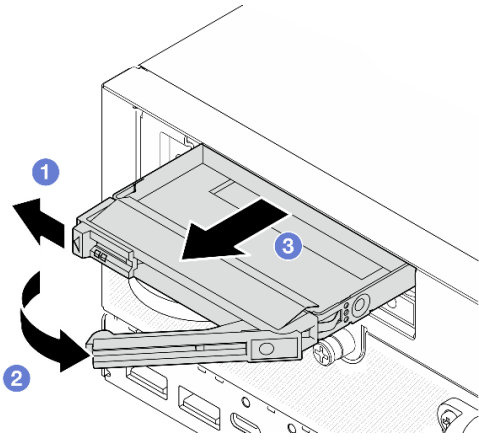
図 78. ドライブ・フィラーの取り外し
