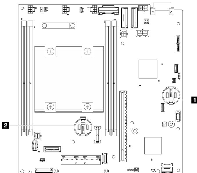
図 117. システム・ボード上の CMOS バッテリーの位置
