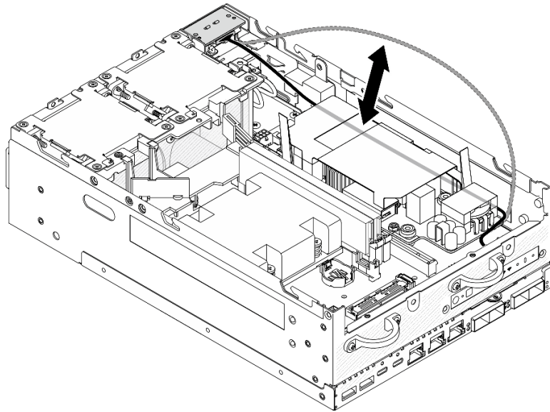
図 137. 信号ケーブルの配置
