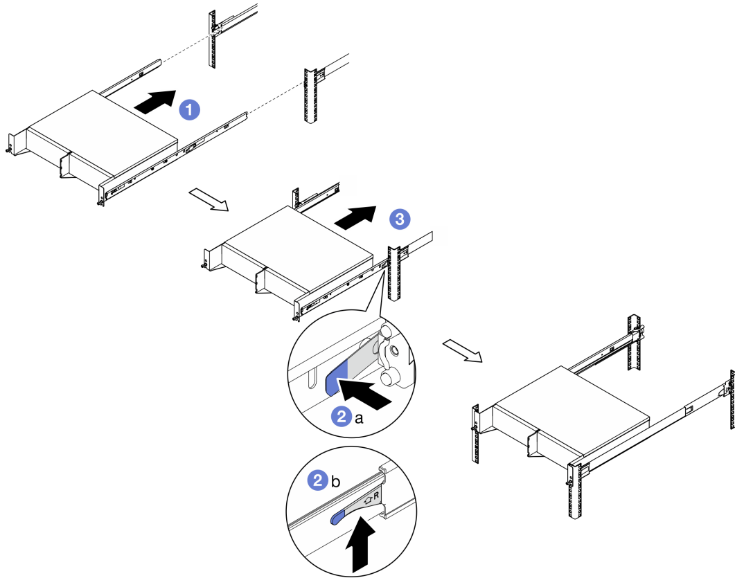
図17. ラックへのエンクロージャーの取り付け
