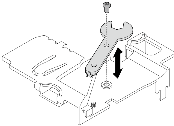
図 320. レンチの保管
