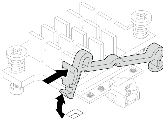
図94. ケーブル・ホルダーの持ち上げ
