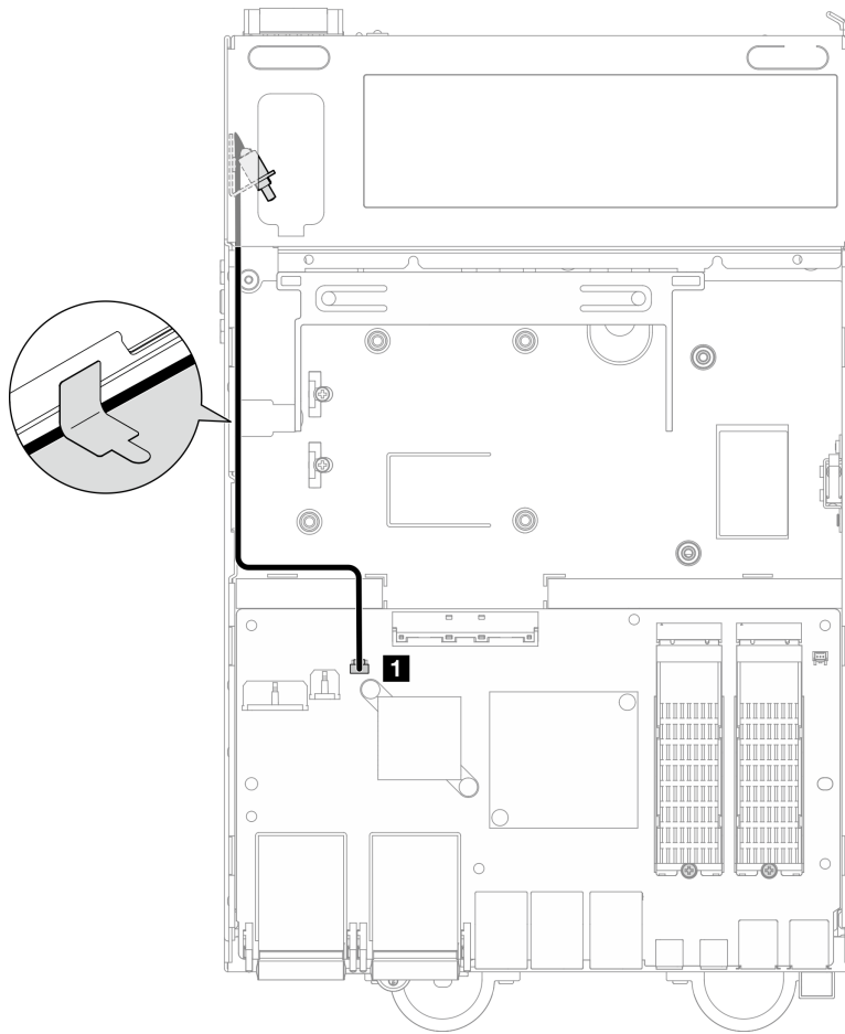
図 170. ロック位置スイッチのケーブル配線
