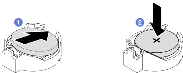
図 121. CMOS バッテリーの取り付け
