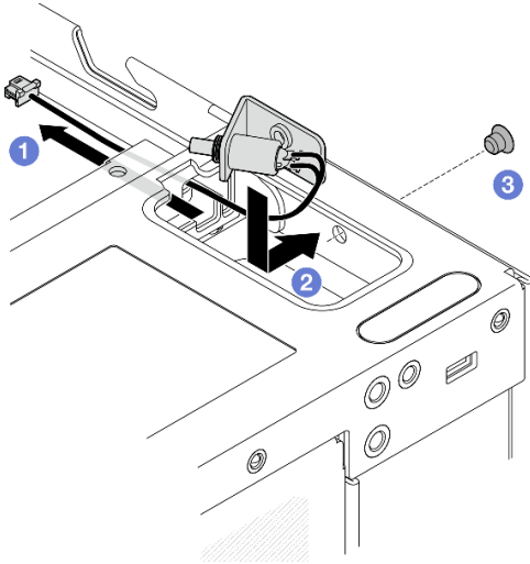
図 169. ケーブル付きロック位置スイッチの取り付け
