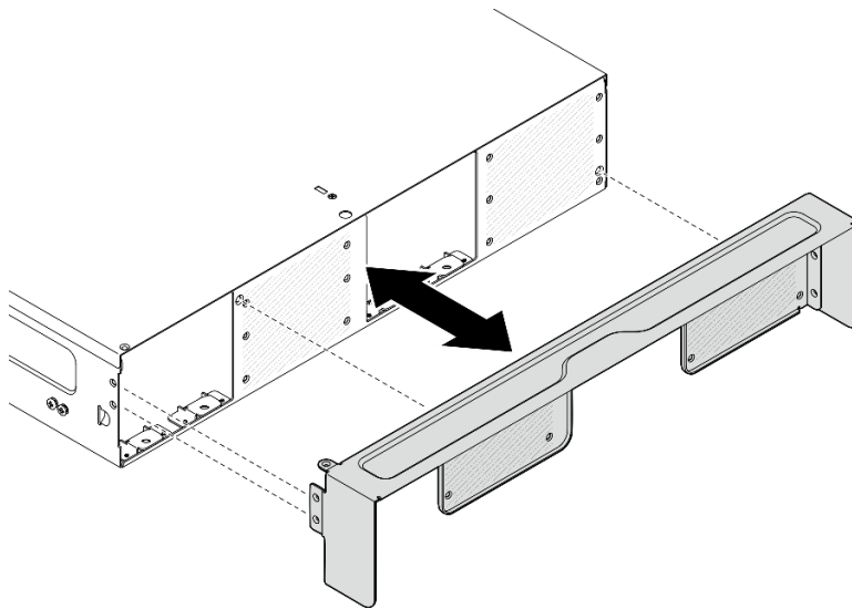
図11. 配送用ブラケットの取り外し
