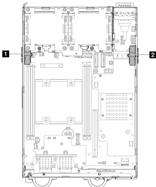
図 323. SMA アセンブリーの位置
