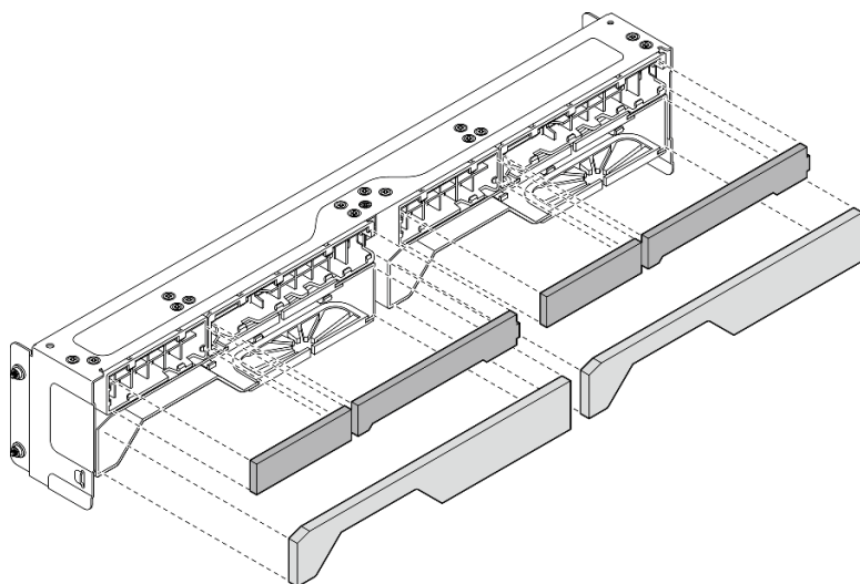
図 69. 防塵フィルターの取り付け
