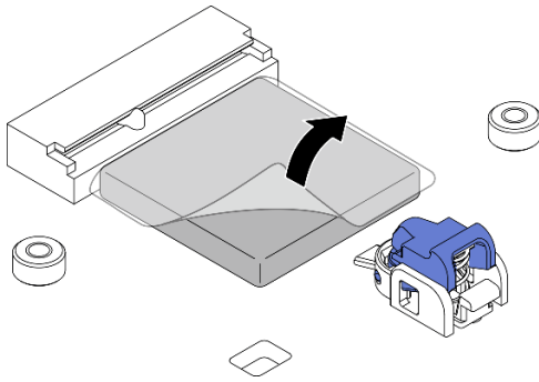
図 286. サーマル・パッドからのフィルムの取り外し
