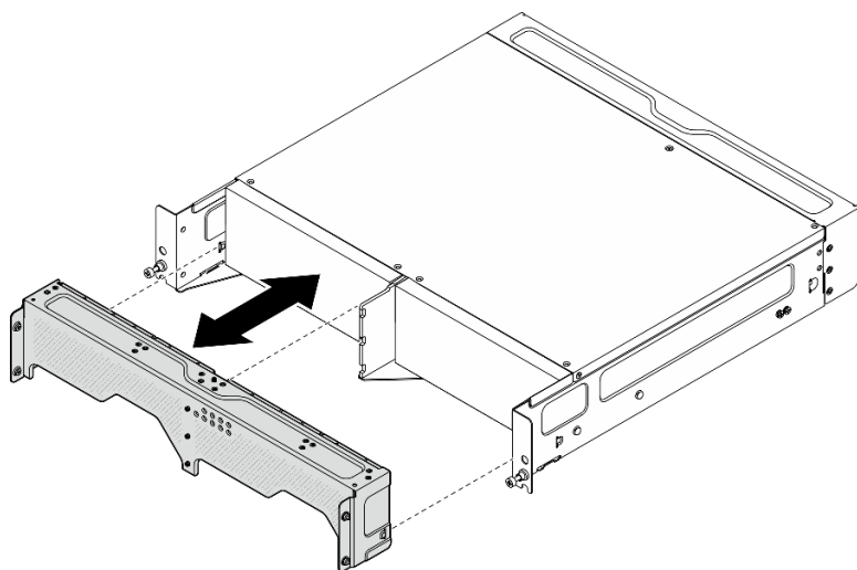
図 70. 配送用ブラケットの取り付け
