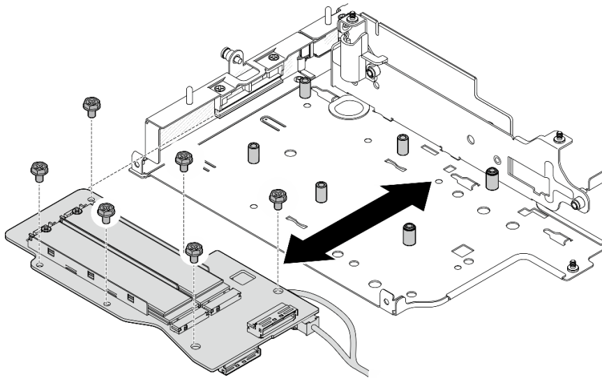
図 248. M.2 アダプターの取り付け
