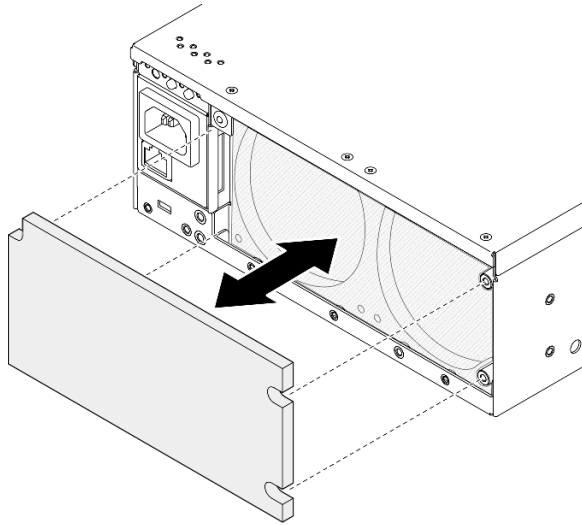
図 74. 防塵フィルターの取り付け
