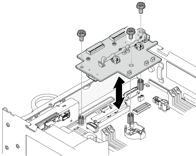
図 283. ワイヤレス・アダプターの取り外し
