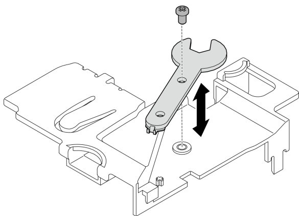
図111. レンチの保管
