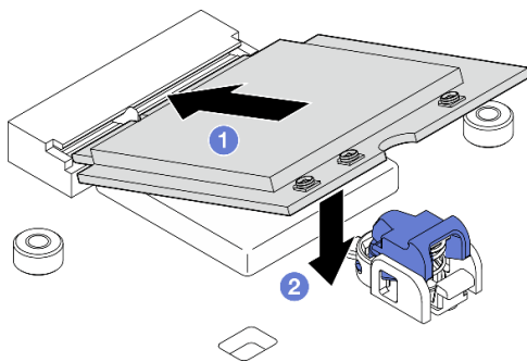
図 287. WLAN/Bluetooth モジュールの取り付け
