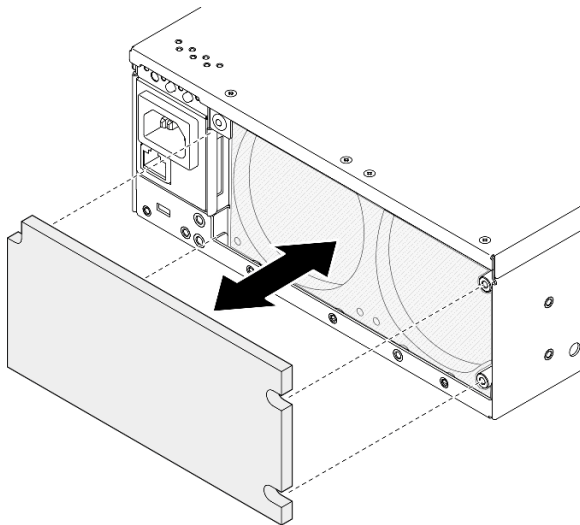
図 73. 防塵フィルターの取り外し
