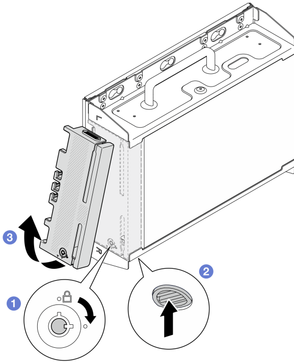
図 50. セキュリティー・ベゼルの取り外し
