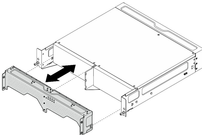
図3. 配送用ブラケットの取り外し
