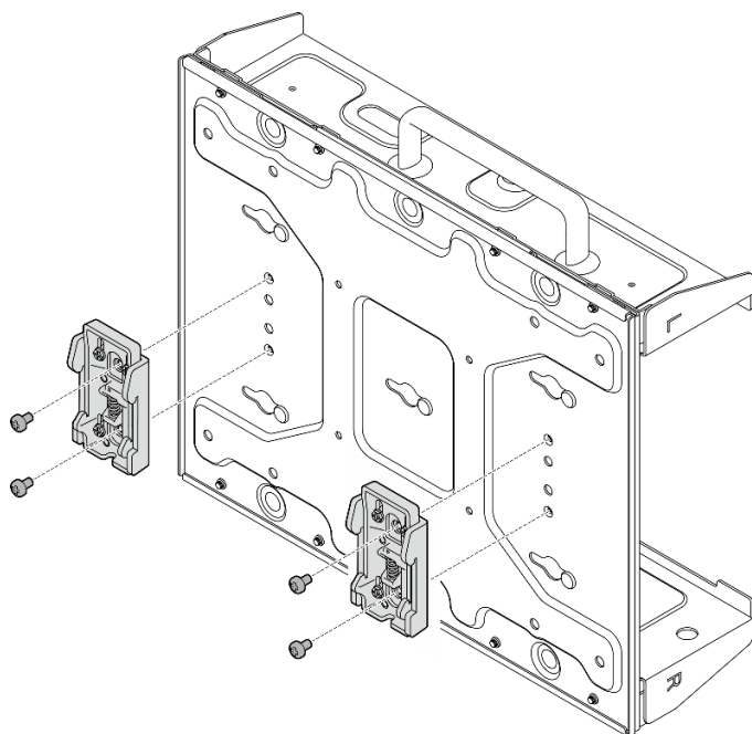
図 53. DIN レール・クリップの取り外し
