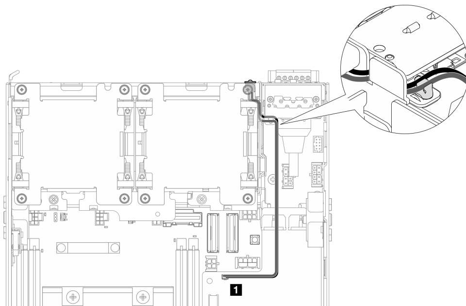
図215. PMB LED ケーブル
