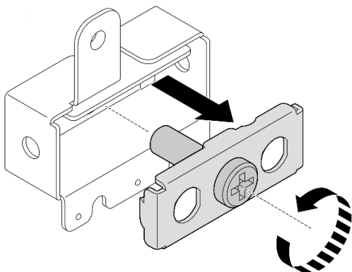
図 324. ブラケットの取り外し
