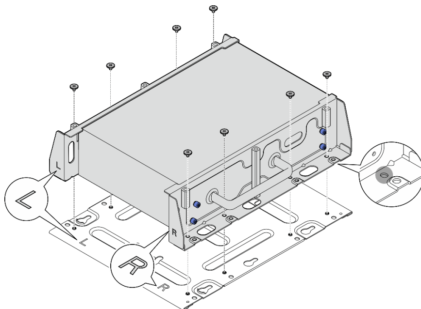
図 54. 下部プレートの取り外し
