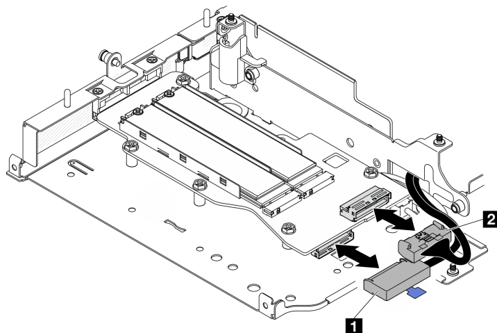
図 249. 信号ケーブルの取り外し
