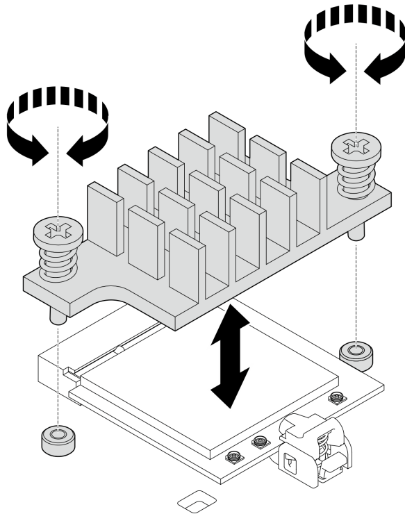
図 289. WLAN/Bluetooth モジュール・ヒートシンクの取り付け
