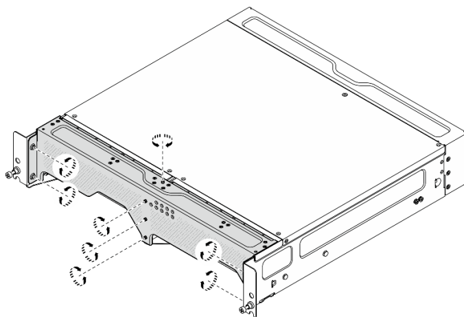
図2. ねじを緩める
