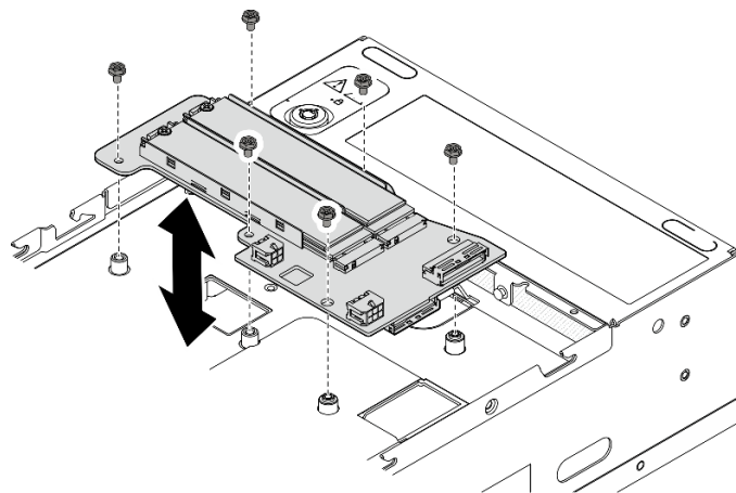
図 113. 下部の M.2 ケーブル接続アダプターの取り外し
