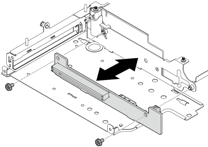
図 254. ライザー・カードの取り付け
