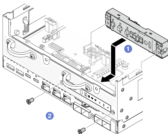
図 131. 前面オペレーター・パネルの取り付け
