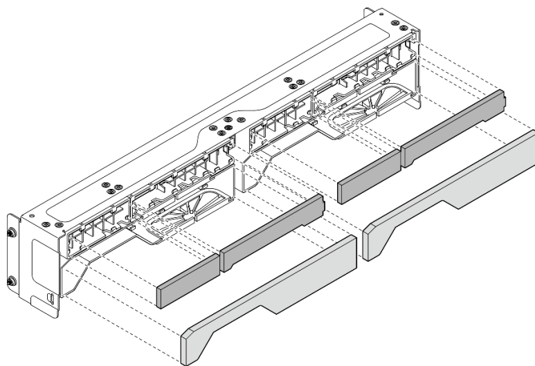
図 68. 防塵フィルターの取り外し
