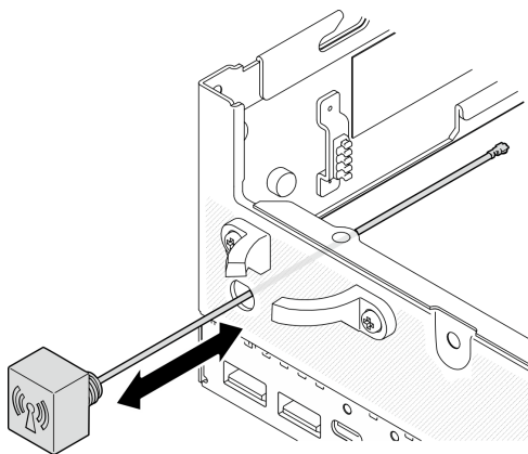
図 103. Bluetooth アンテナの取り付け
