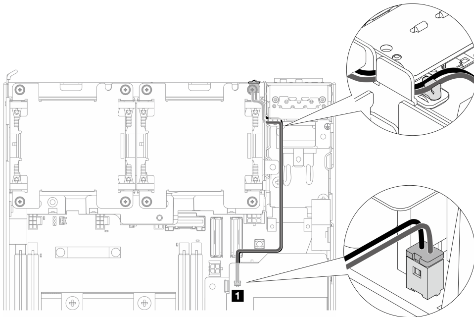
図 197. 内部パワー・サプライ・ユニット (AC PMB) に接続する PMB 状況 LED ケーブル
