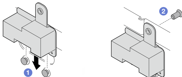
図321. SMA フィラーの取り付け
