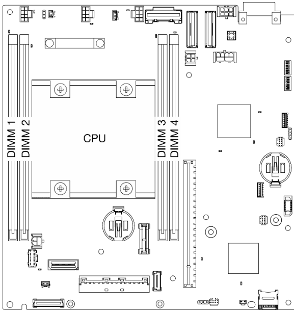
図1. メモリー・モジュールおよびプロセッサのレイアウト
