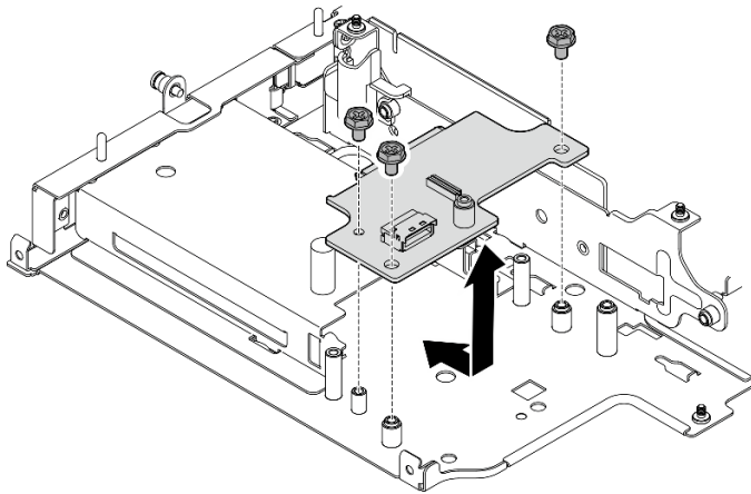
図 252. バックプレーン1の取り付け
