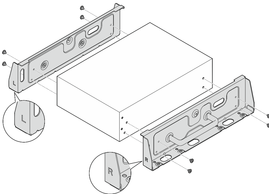
図32. ねじを緩めてサイド・ブラケットを取り外す
