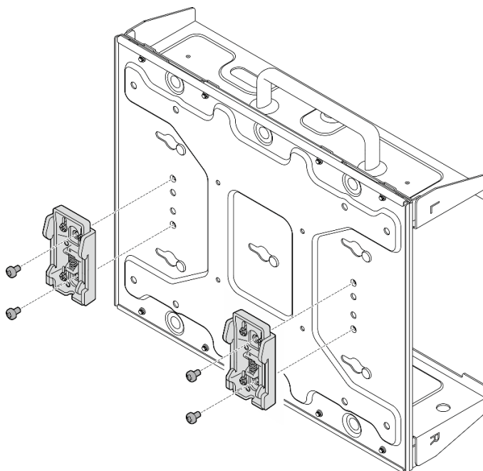
図 63. DIN レール・クリップの取り付け
