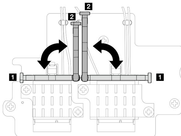
図108. ケーブル・ホルダーの回転
