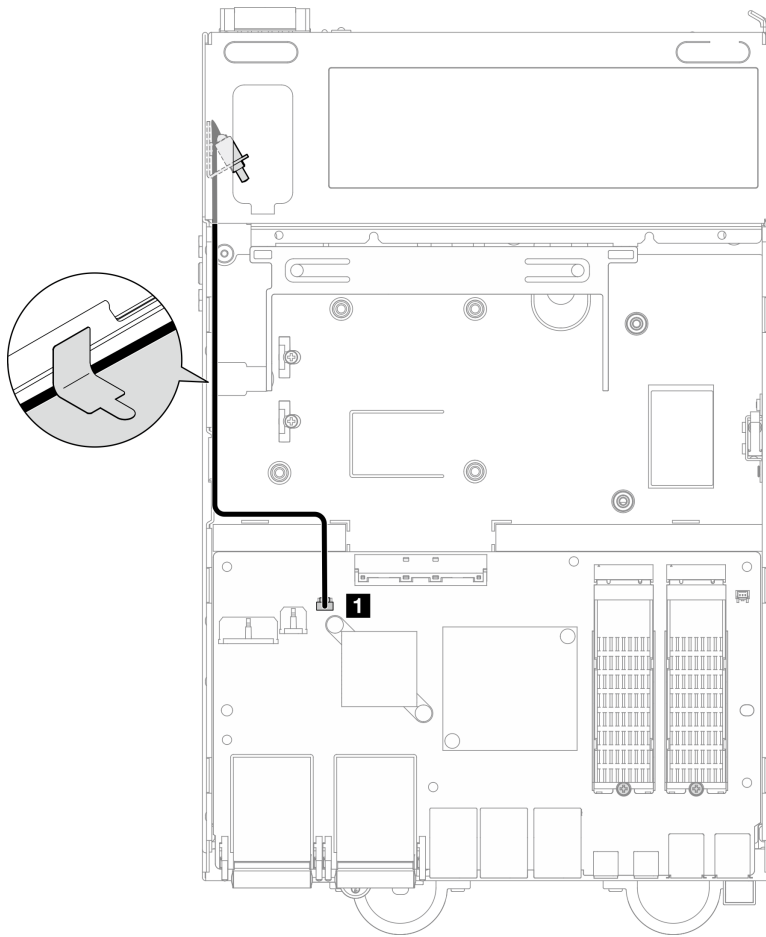
図 167. ロック位置スイッチのケーブル配線
