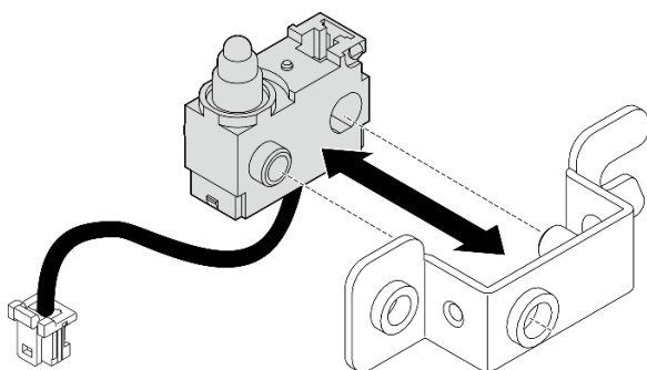
図 144. ブラケットからの侵入検出スイッチの分離
