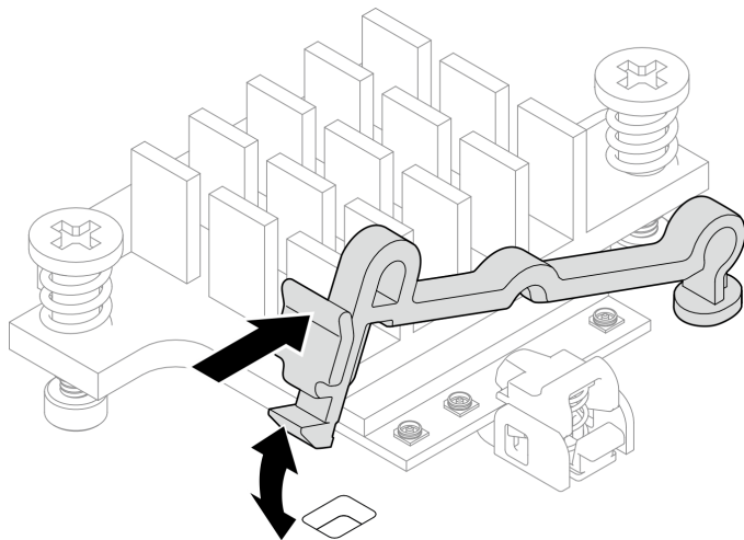
図333. ケーブル・ホルダーの挿入
