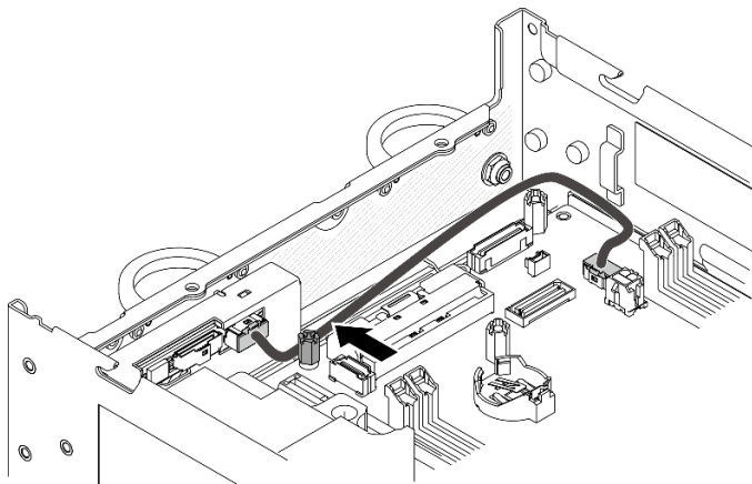
図341. 前面オペレーター・パネルのケーブル配線
