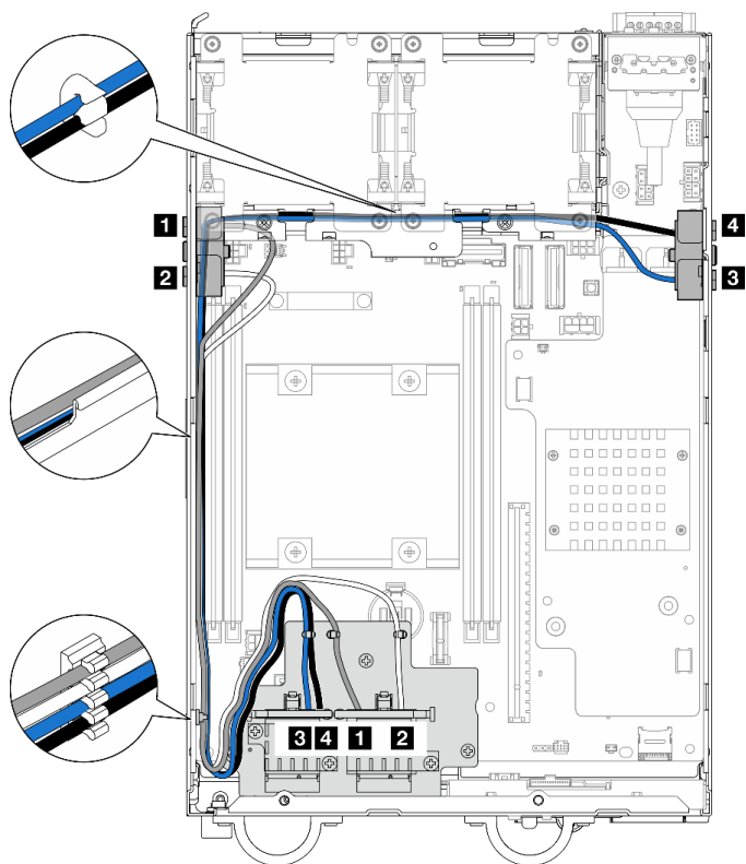
図 327. SMA アセンブリーのケーブル配線
