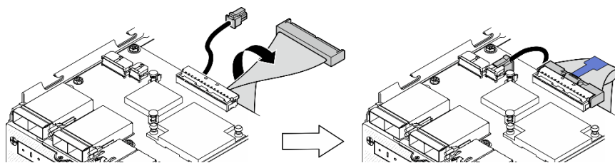
図 161. I/O ボード・ケーブルの接続
