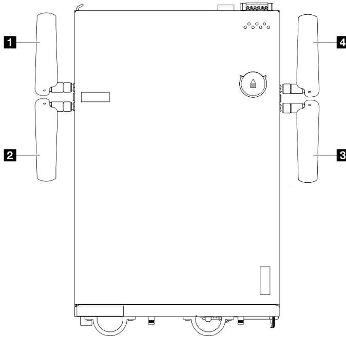
図 295. WLAN アンテナの位置
