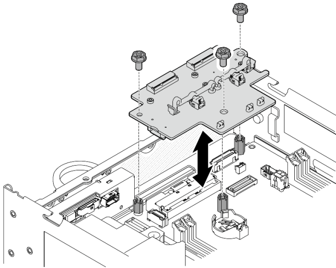
図 284. ワイヤレス・アダプターの取り付け
