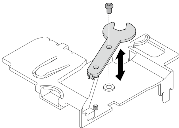
図 298. レンチの取り外し
