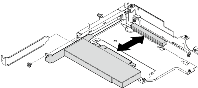
図 255. PCIe アダプターの取り付け
