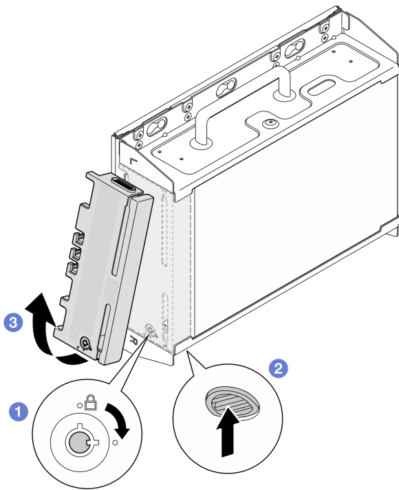
図 26. セキュリティー・ベゼルの取り外し
