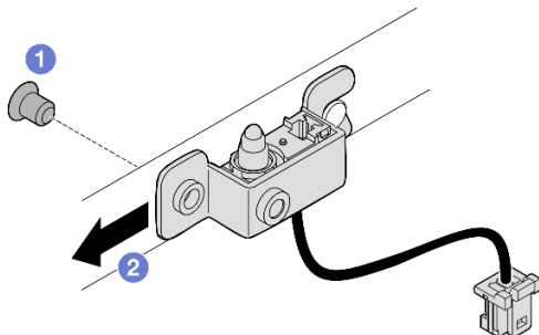
図 143. ケーブル付き侵入検出スイッチ・ケーブルの取り外し
