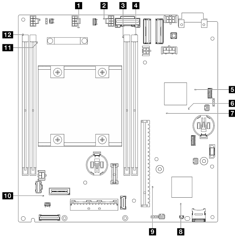
図 351. システム・ボード LED
