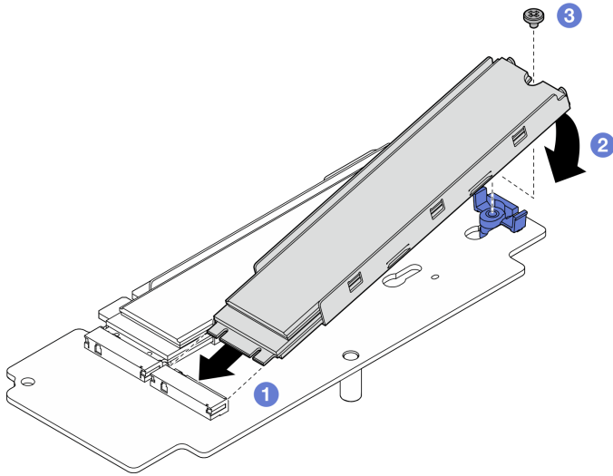
図 241. M.2 ドライブの取り付け
