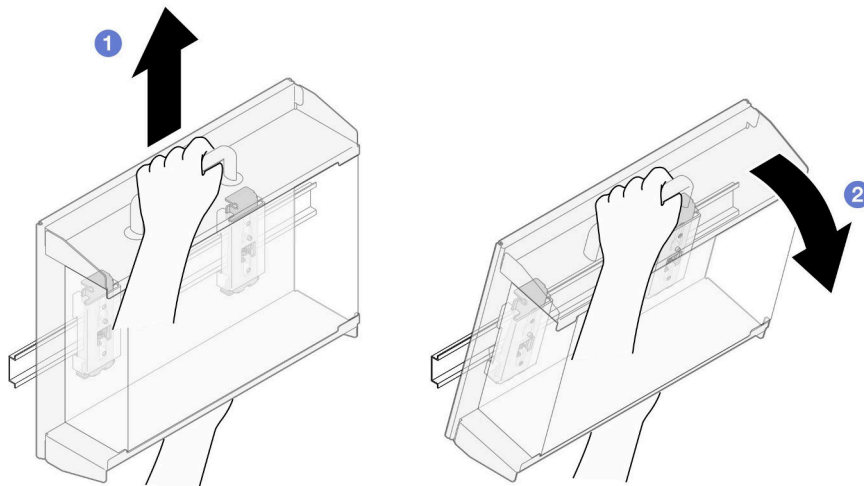
図 51. ノード・スリーブの取り外し
