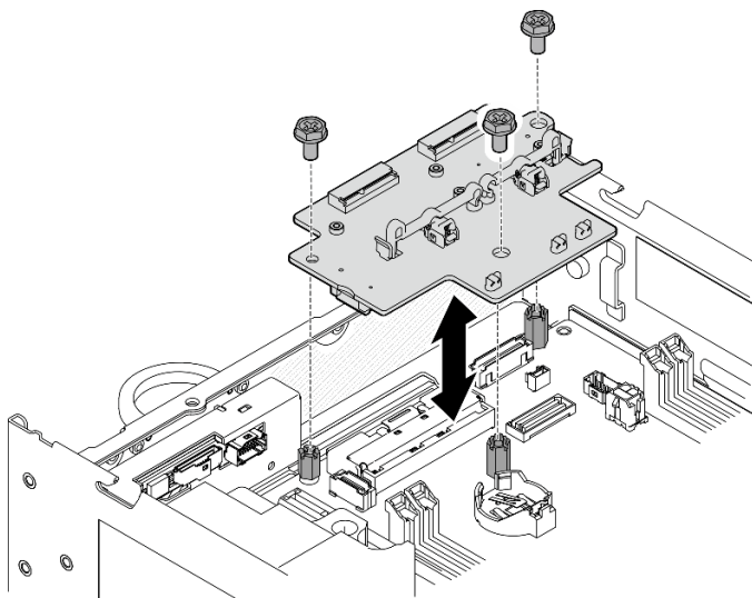
図110. ワイヤレス・アダプターの取り付け
