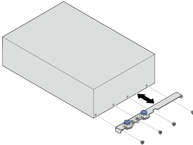
図20. エンクロージャー・ブラケットの取り付け
