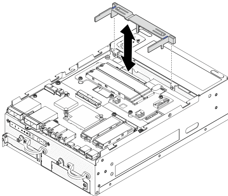
図83. エアー・バッフルの取り付け
