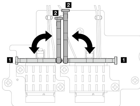
図 279. ケーブル・ホルダーの回転
