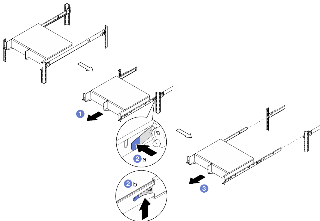
図8. ラックからのエンクロージャーの取り外し
