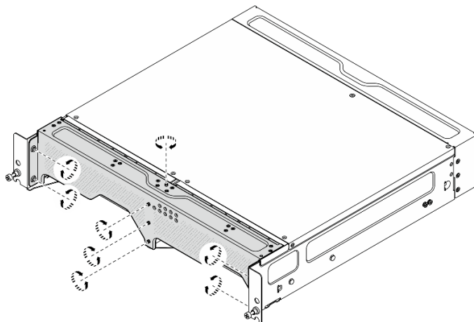
図 25. ねじを締める
