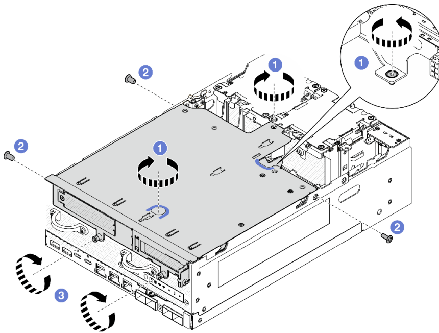
図265. ライザー・アセンブリーの固定
