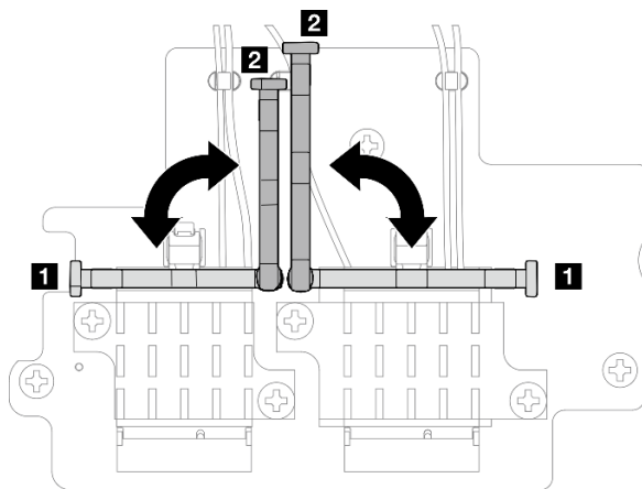
図315. ケーブル・ホルダーの回転
