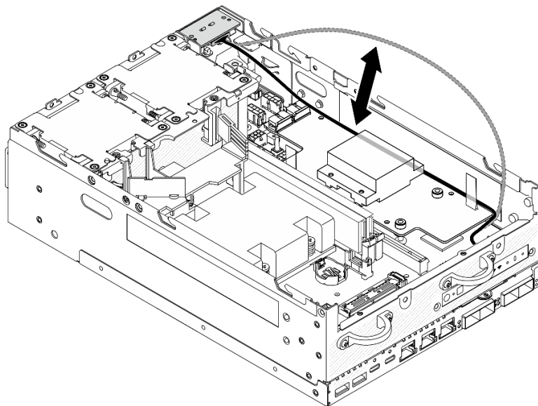
図 207. 信号ケーブルの配置
