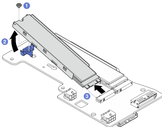
図226. M.2 ドライブの取り外し
