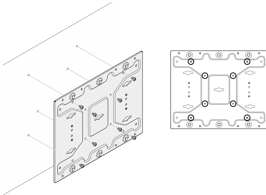
図44. 壁掛け用プレートの取り付け
