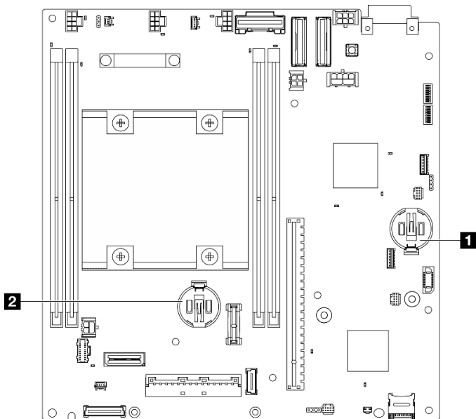
図 120. システム・ボード上の CMOS バッテリーの位置
