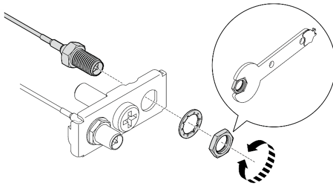
図319. ブラケットからケーブルを緩める
