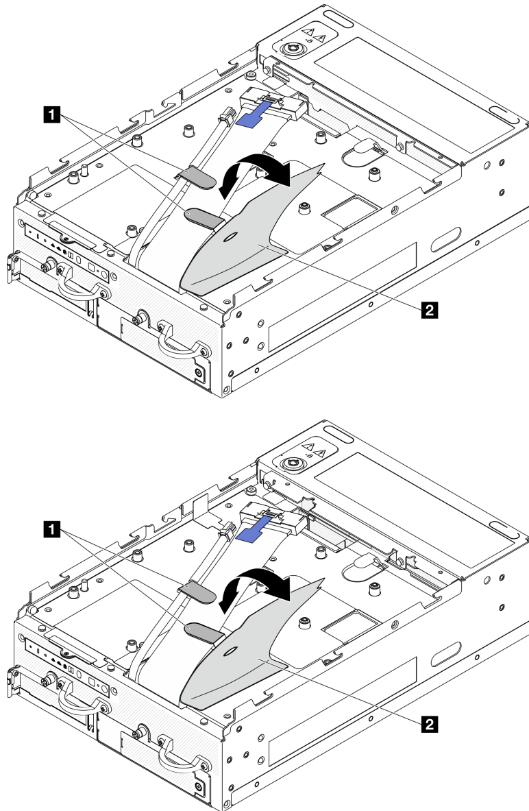
図159. I/O ボードのケーブル配線
