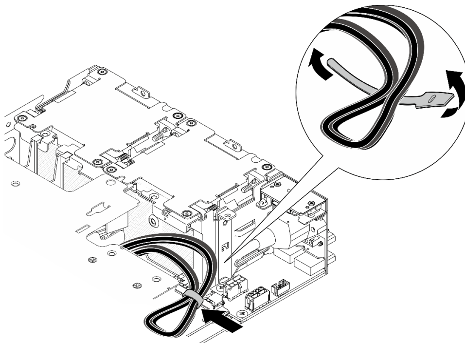
図 262. ライザー・アセンブリーのケーブル配線
