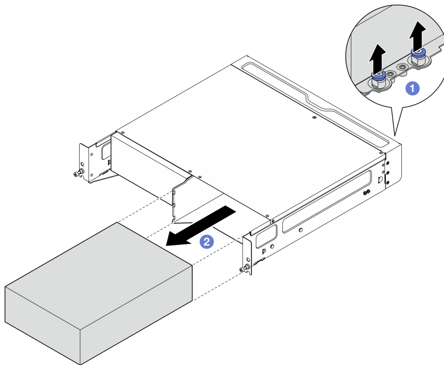
図4. ノードの取り外し
