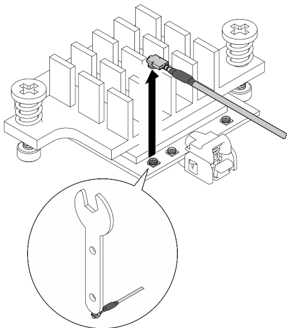
図314. ケーブルの取り外し
