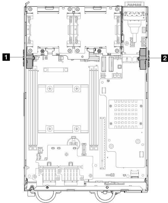
図 297. SMA アセンブリーの位置
