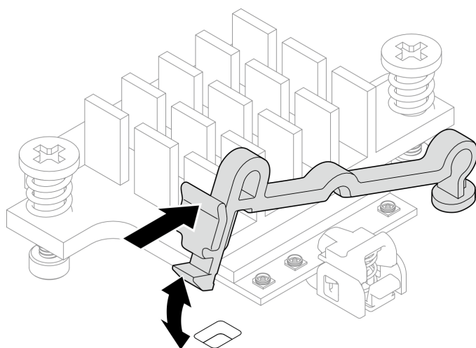
図109. ケーブル・ホルダーの挿入
