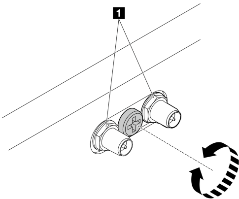
図 337. SMA コネクタの延長
