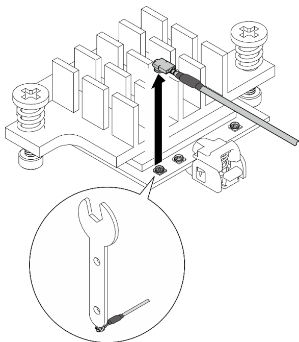
図96. ケーブルの取り外し
