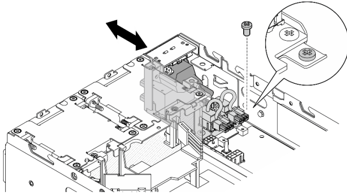
図 202. DC PIB モジュールの取り外し
