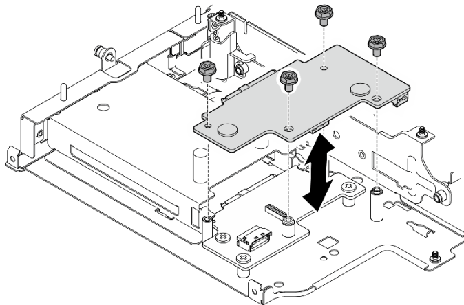
図 253. バックプレーン 2 の取り付け
