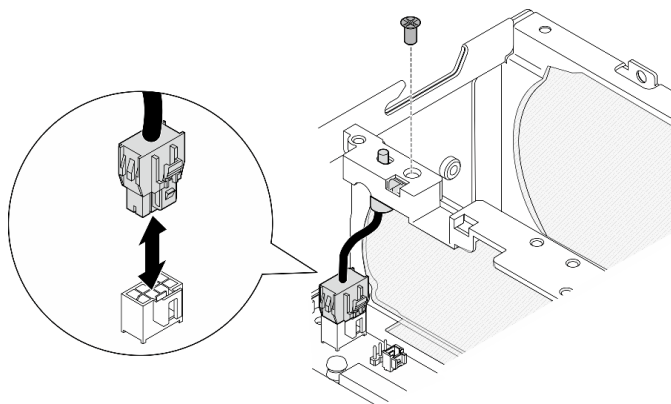
図 125. ファン方向スイッチの取り付け
