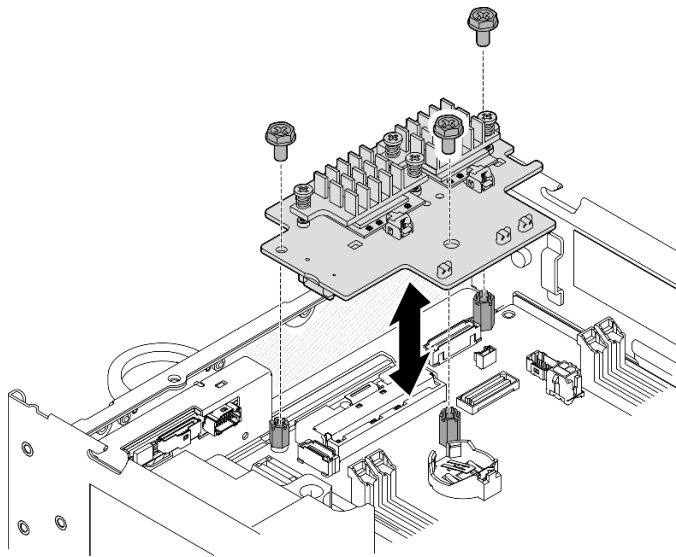
図93. ワイヤレス・アダプターの持ち上げ
