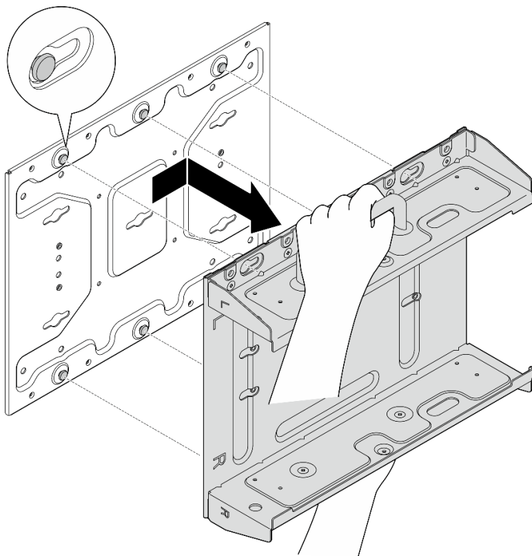
図 28. ノード・ブラケットの取り外し
