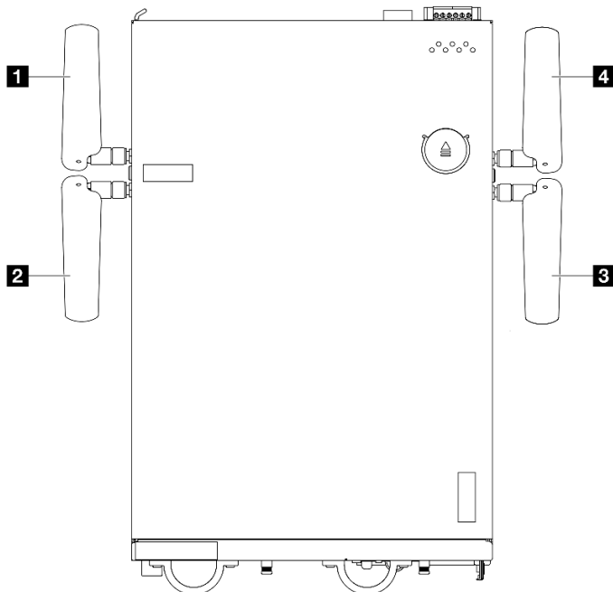
図 352. WLAN アンテナの位置
