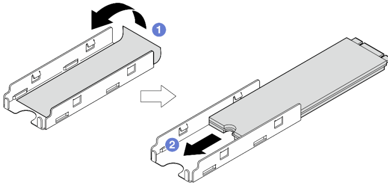
図174. M.2 ドライブの取り付け
