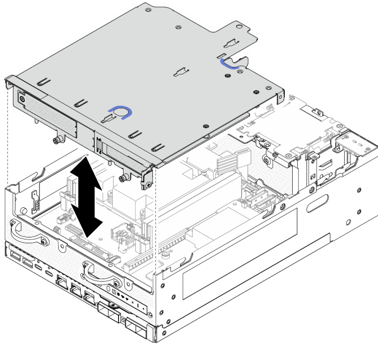
図260. ライザー・アセンブリを下げる
