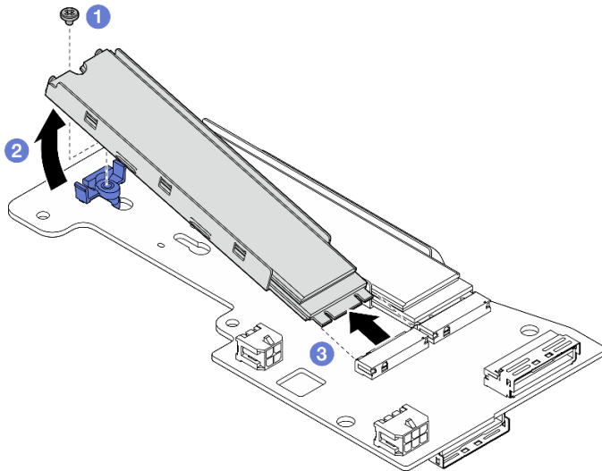
図 112. M.2 ドライブの取り外し
