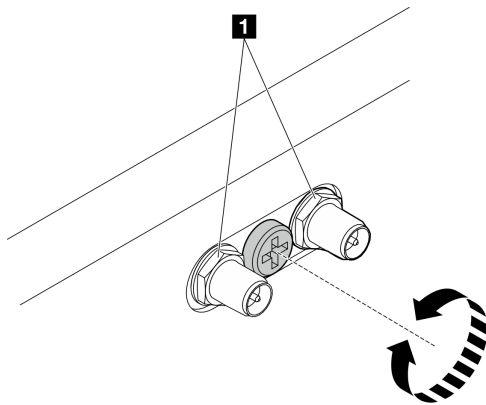
図 19. SMA コネクターの短縮
