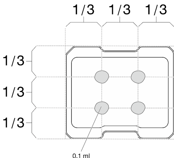
図 218. 熱伝導グリースの適切な形
