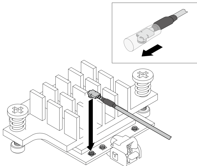
図 107. ケーブルの接続
