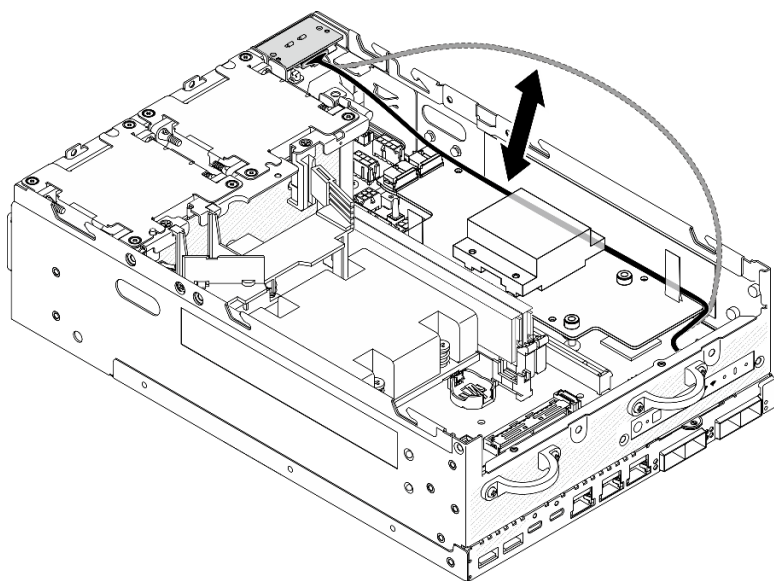
図 211. 信号ケーブルの配置
