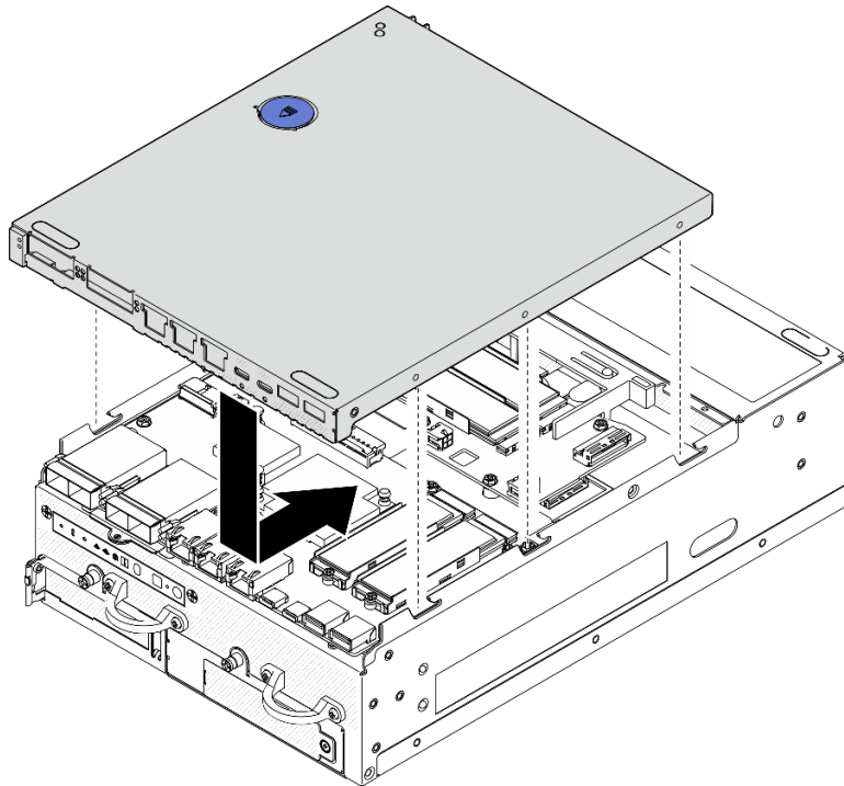
図194. 下部カバーの取り付け
