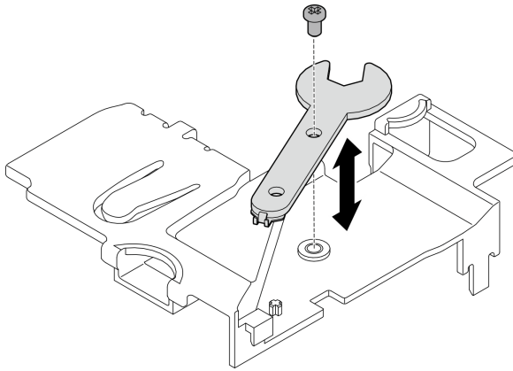
図 335. レンチの保管
