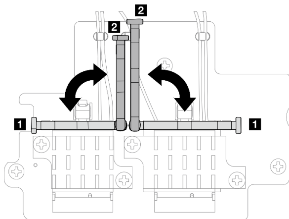
図 106. ケーブル・ホルダーの回転
