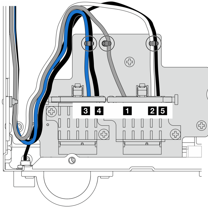
図 290. ワイヤレス・アダプターのケーブル配線
