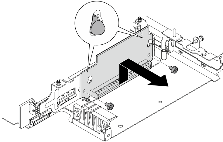
図 240. ライザー・カードの取り外し
