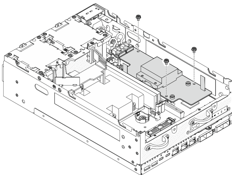
図 209. ねじを緩める
