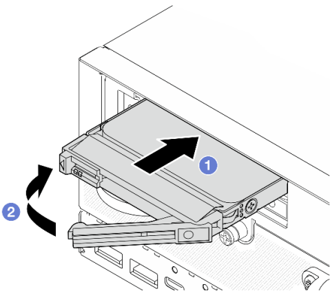
図 79. 7 mm ドライブの取り付け
