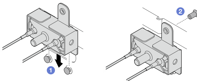
図 326. SMA アセンブリーの取り付け
