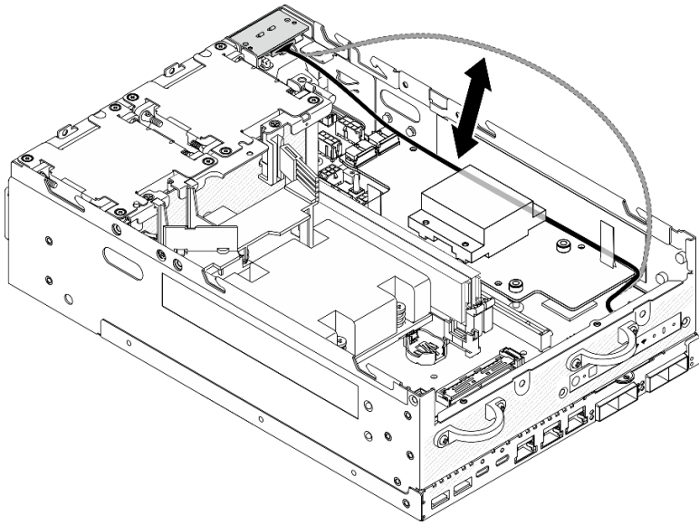
図216. 信号ケーブルの配置
