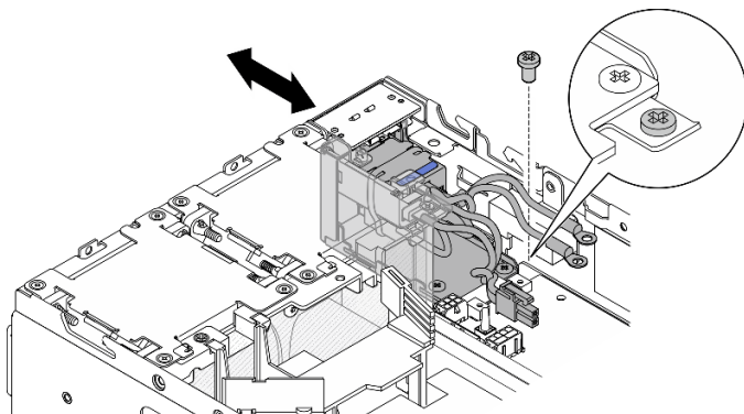
図 203. AC PIB モジュールの取り外し
