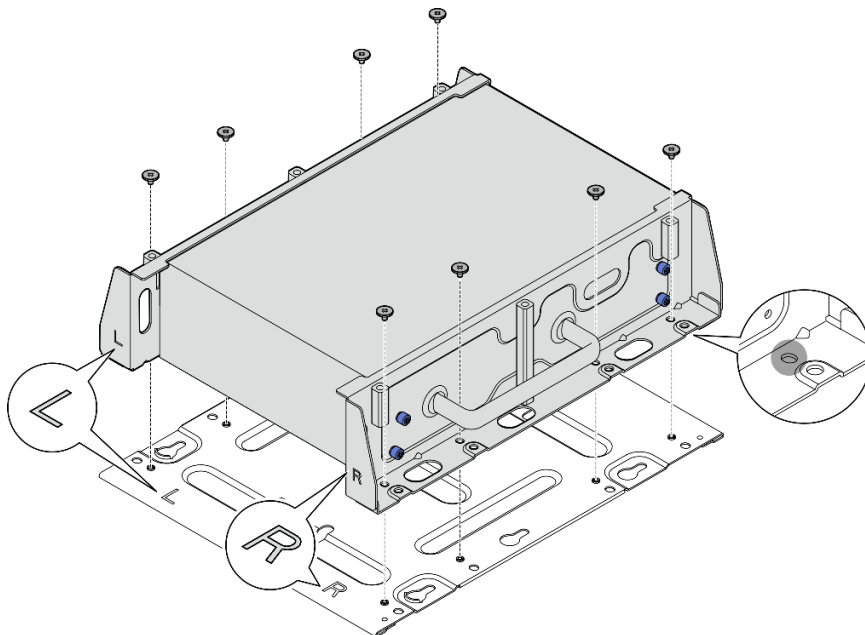
図31. 下部プレートの取り外し
