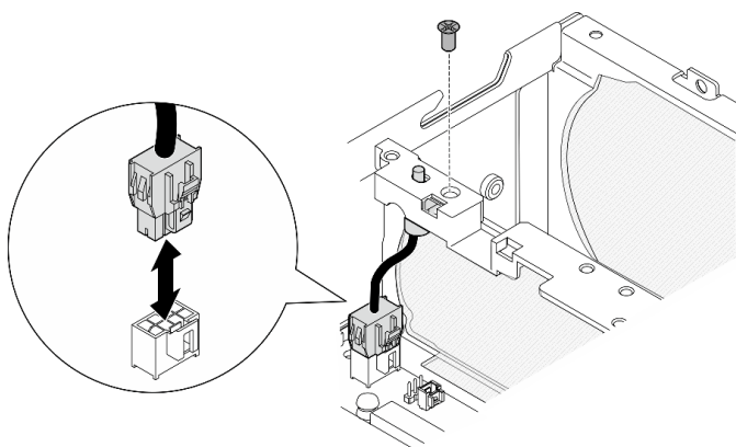
図 122. ファン方向スイッチの取り外し
