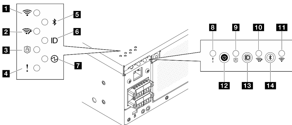
図 350. 背面オペレーター・パネル LED
