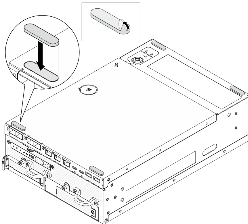
図 271. ラバー・フィートの取り付け
