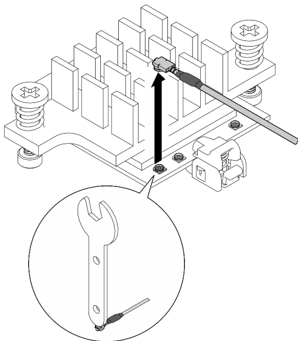
図 280. ケーブルの取り外し
