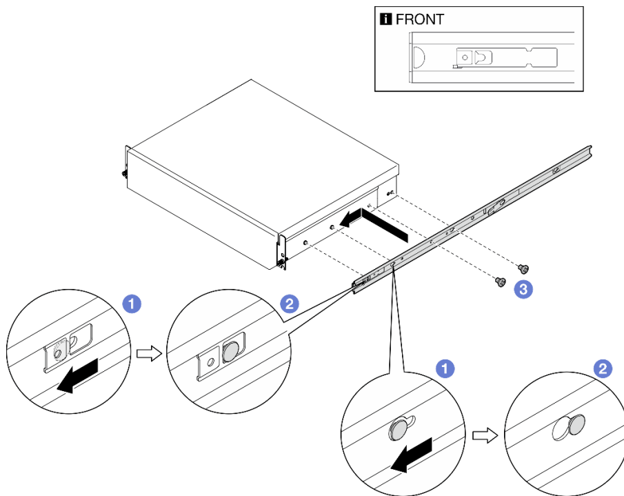
図 16. 内側レールの取り付け
