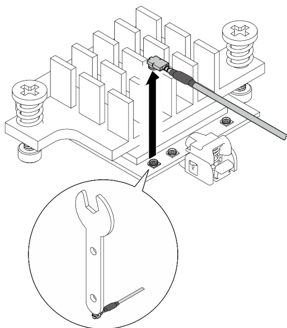
図 303. ケーブルの取り外し
