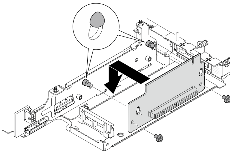
図 242. ライザー・カードの取り付け
