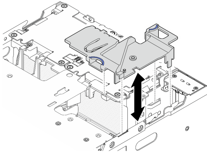
図84. エアー・バッフルの取り外し
