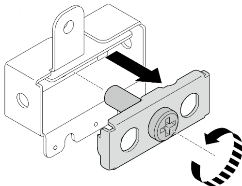
图 324. 卸下支架
