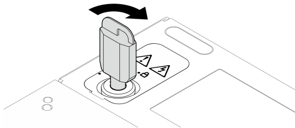
图 186. 锁定钥匙锁
