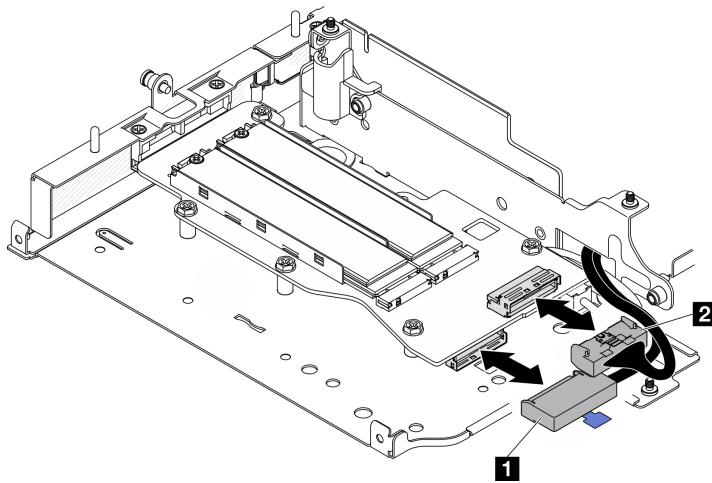
图 249. 拔下信号线缆
