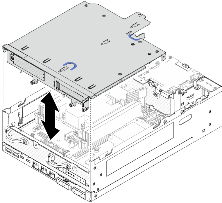
图 266. 下放转接卡组合件
