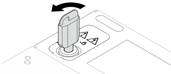
图 193. 解锁钥匙锁
