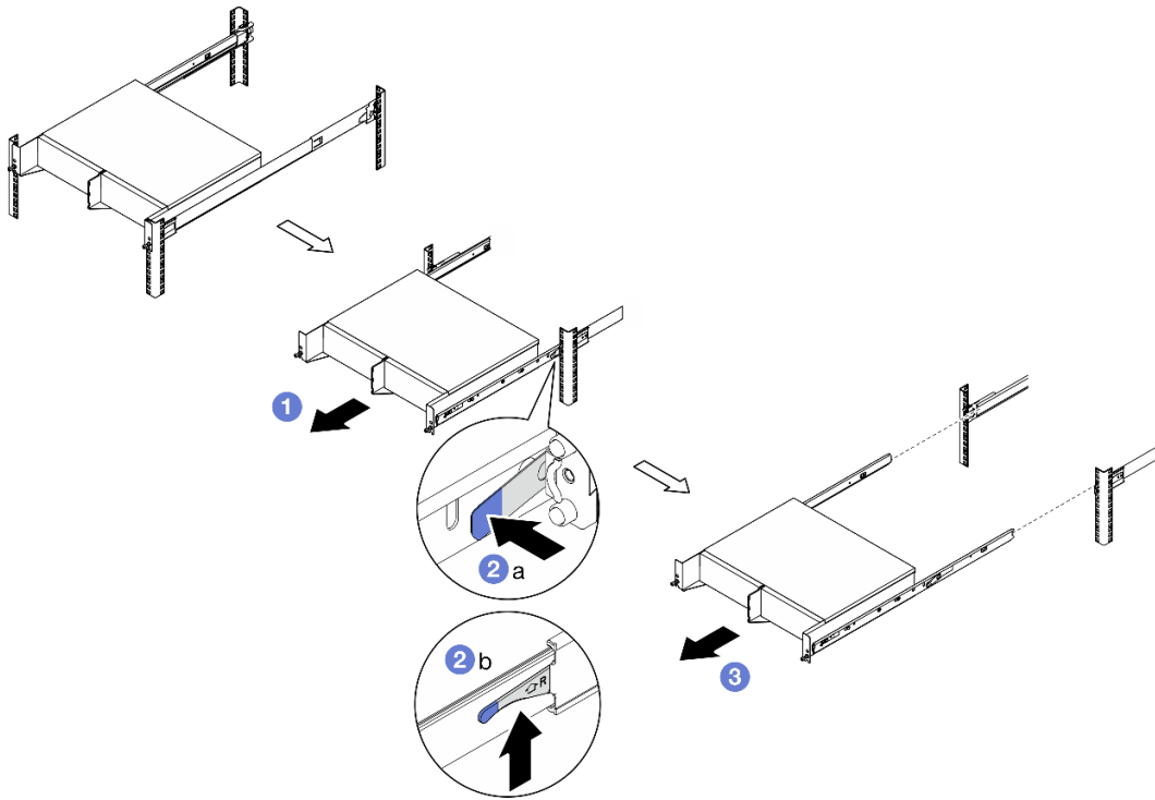
图 8. 从机架上卸下机柜
