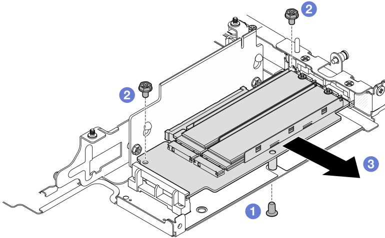
图 236. 卸下 M.2 适配器
