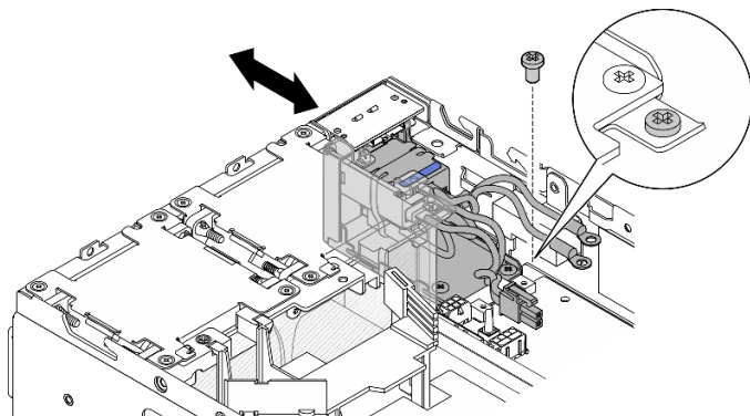
图 206. 安装 PIB 模块
