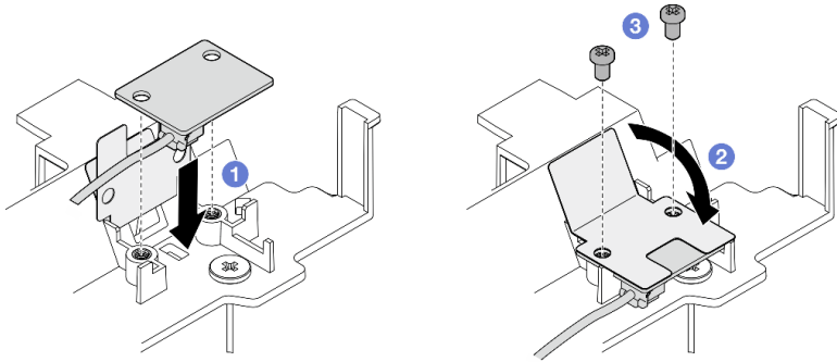
图 90. 安装气流传感器板
