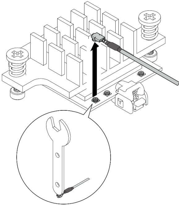
图 314. 拔下线缆
