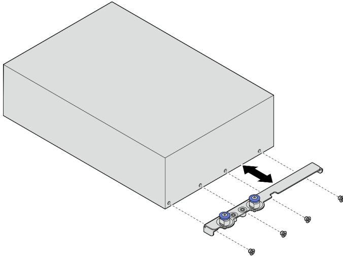
图 20. 安装机柜支架
