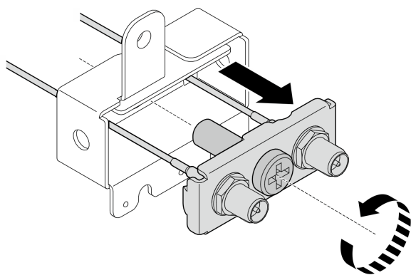
图 307. 卸下支架
