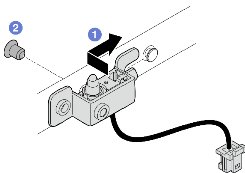
图 146. 安装带线缆的入侵感应开关
