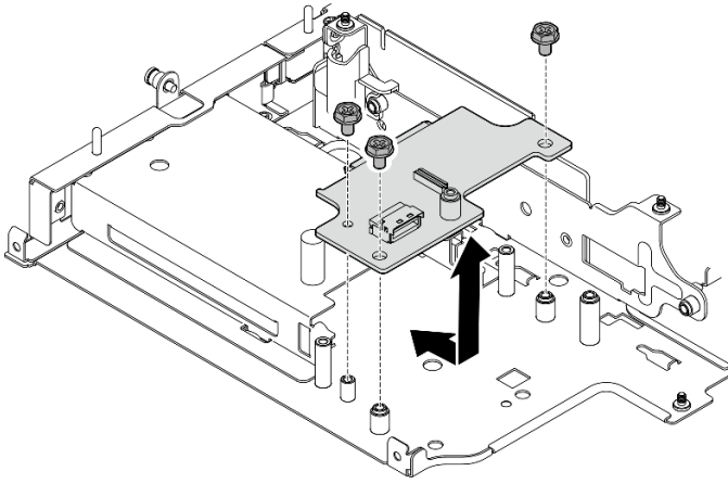
图 252. 安装背板 1
