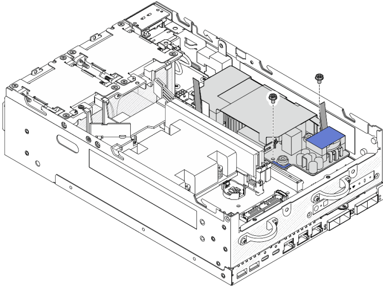
图 135. 拧松螺钉
