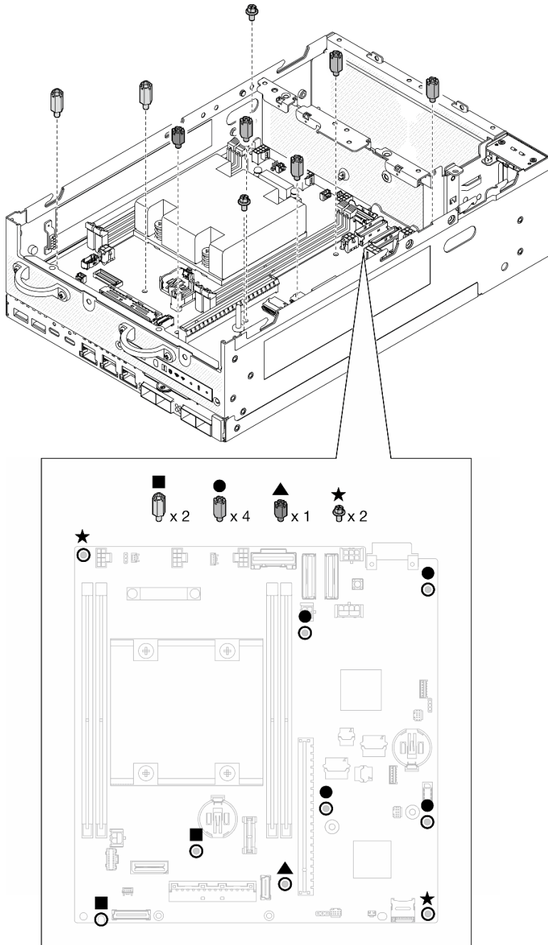
图 275. 主板上的螺钉和支脚
