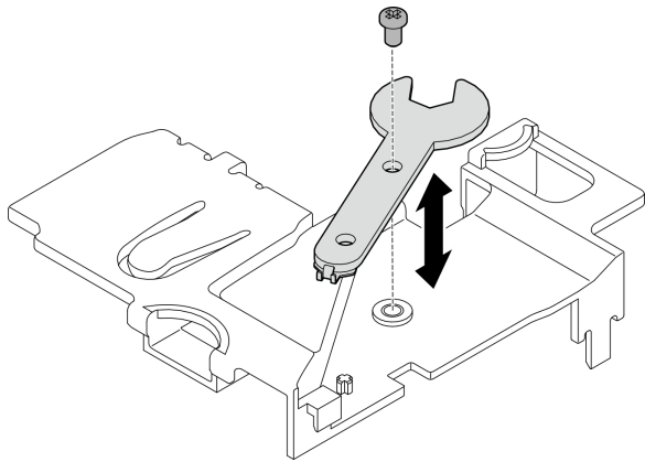
图 309. 存放扳手
