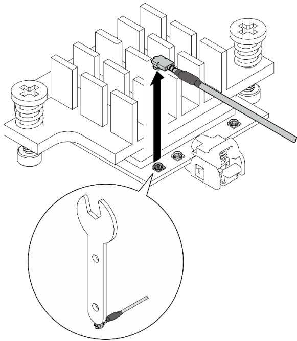
图 280. 拔下线缆
