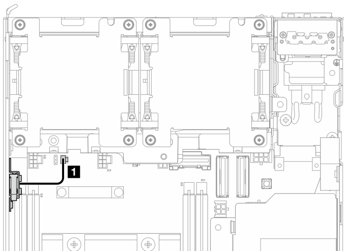
图 147. 顶部入侵感应开关线缆布放
