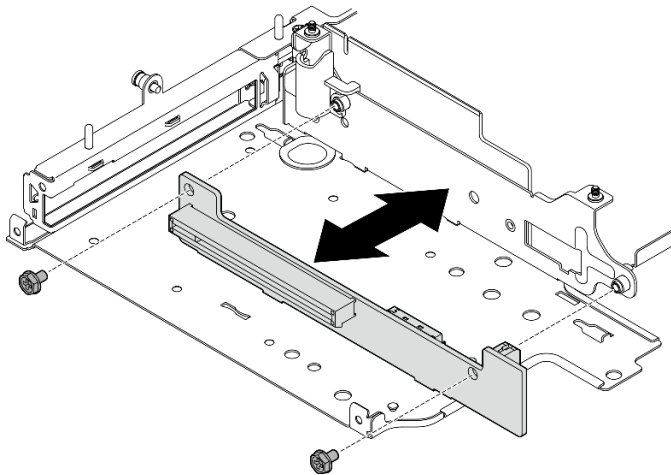
图 228. 卸下转接卡
