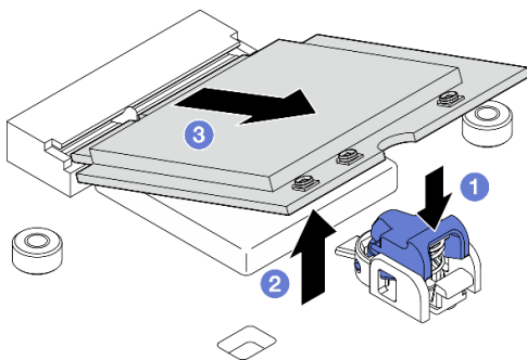
图 282. 卸下 WLAN/蓝牙模块
