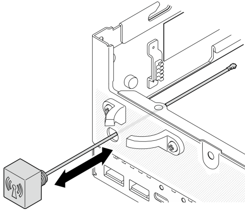
图 100. 卸下蓝牙天线
