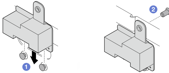
图 321. 安装 SMA 填充件
