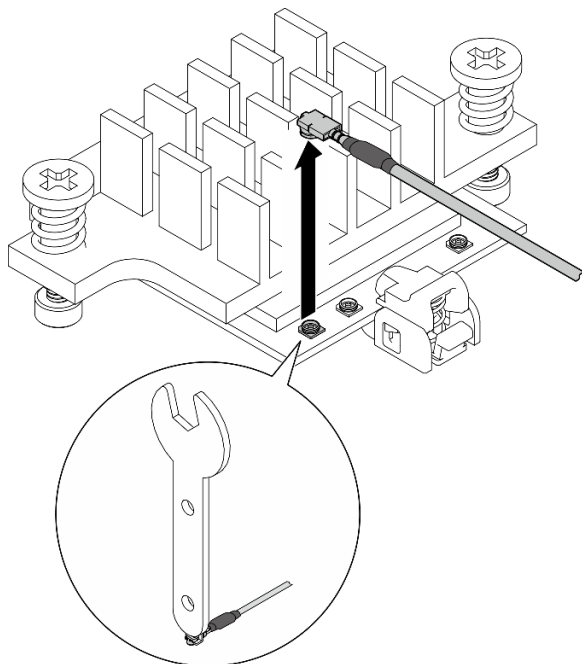
图 96. 拔下线缆
