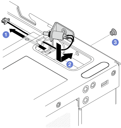
图 169. 安装带线缆的锁定位置开关
