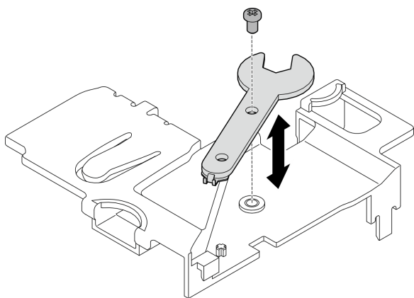
图 102. 取下扳手
