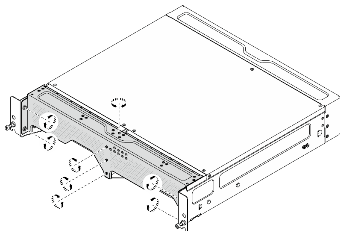
图 25. 拧紧螺钉
