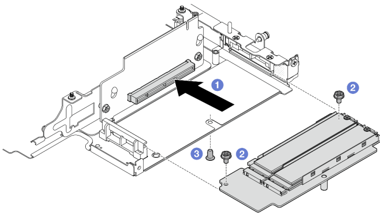
图 243. 安装 M.2 适配器
