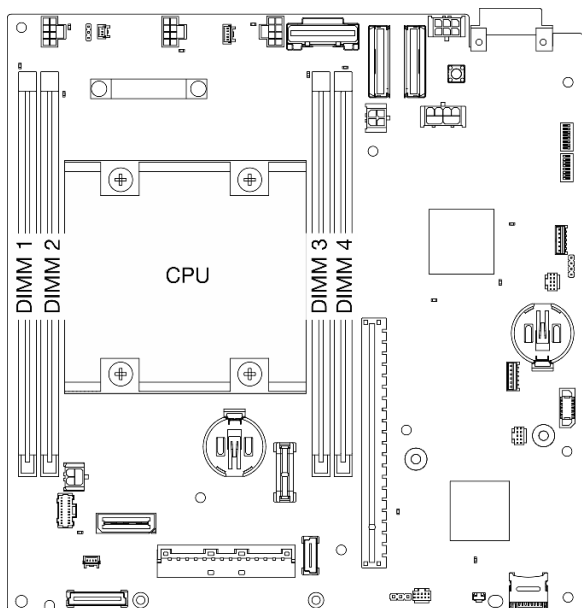
图 1. 内存条和处理器布局
