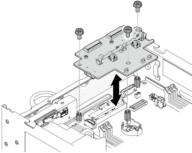
图 283. 卸下无线适配器
