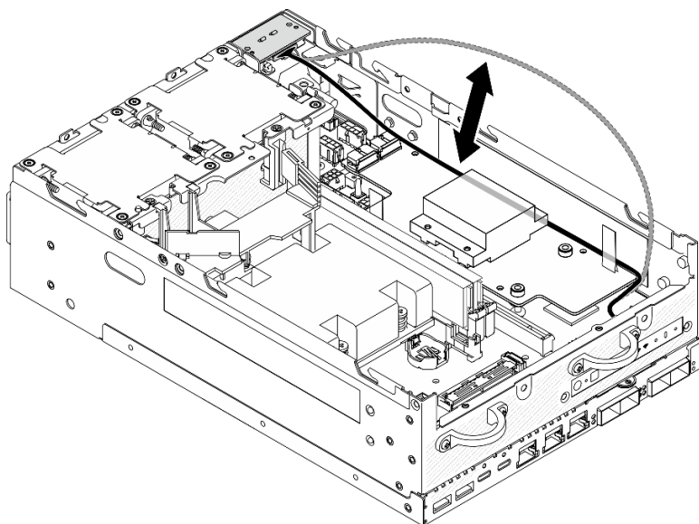
图 211. 放置信号线缆
