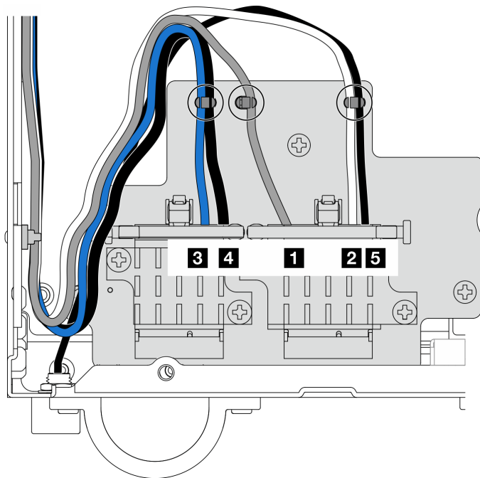
图 294. 无线适配器线缆布放
