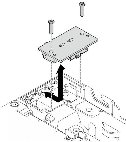
图 221. 安装背面操作员面板
