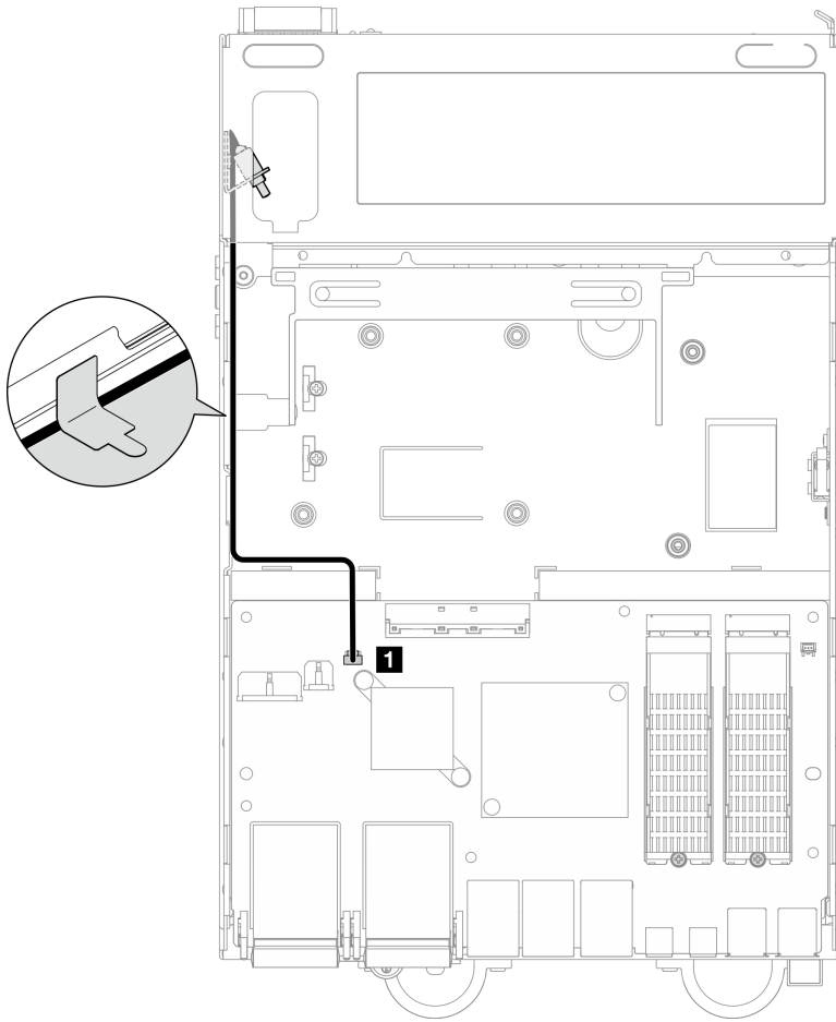
图 167. 锁定位置开关线缆布放
