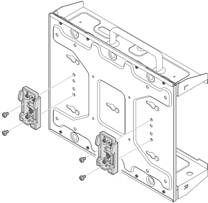
图 53. 卸下 DIN 导轨夹
