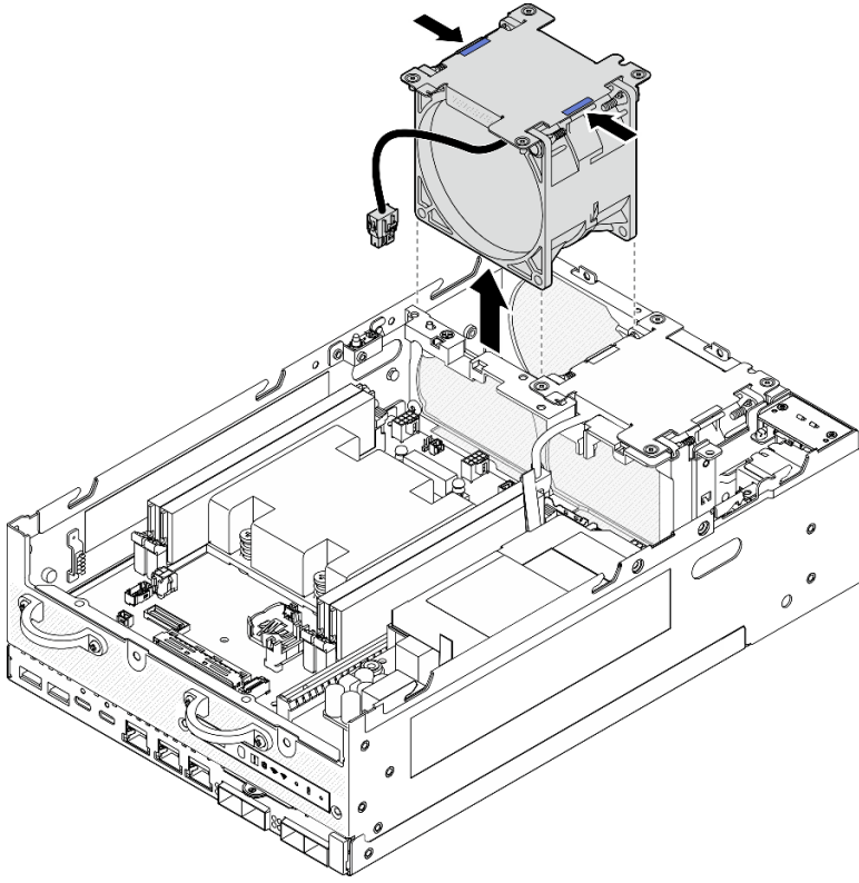
图 127. 卸下风扇模块
