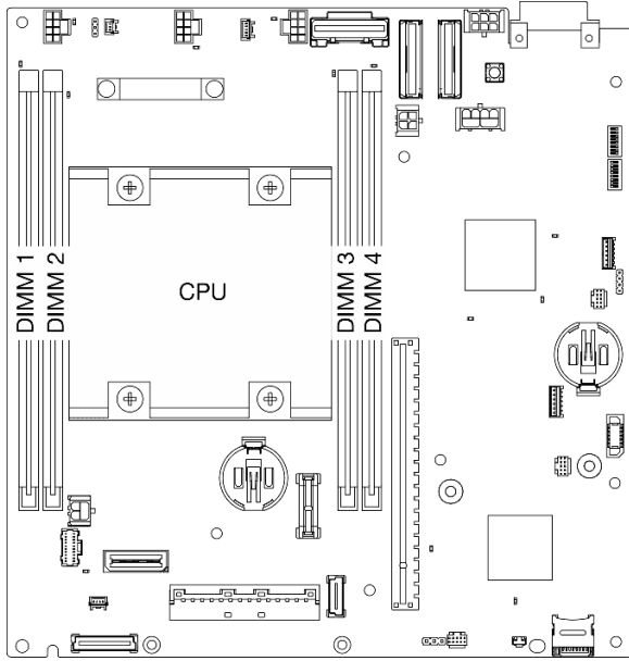
图 179. 内存条和处理器布局
