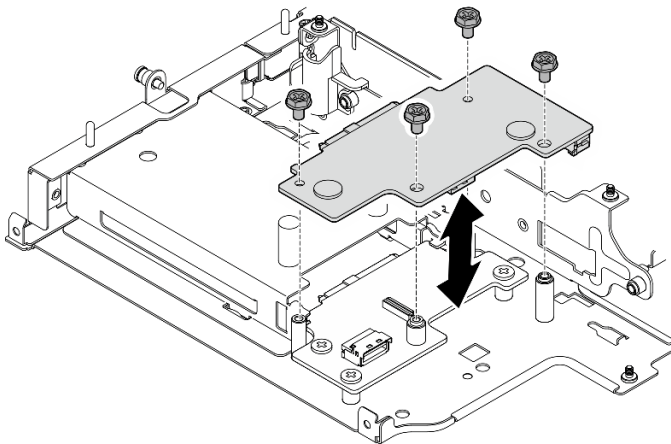
图 253. 安装背板 2
