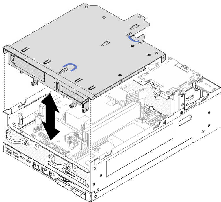
图 260. 下放转接卡组合件
