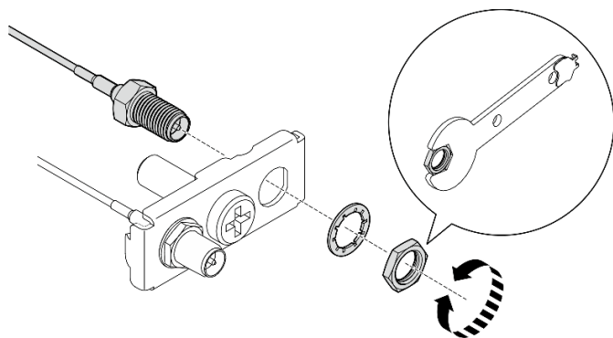
图 308. 从支架上松开线缆
