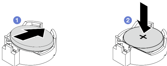
图 121. 安装 CMOS 电池
