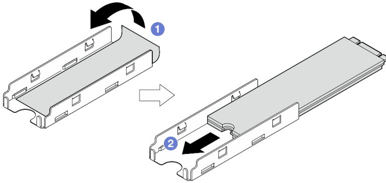
图 174. 安装 M.2 硬盘
