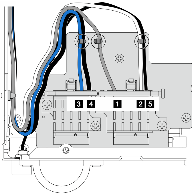
图 343. WLAN 天线和蓝牙天线线缆布放
