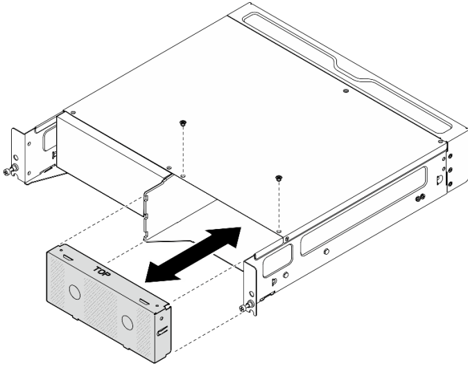
图 5. 安装节点填充件
