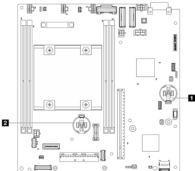
图 120. 主板上的 CMOS 电池位置
