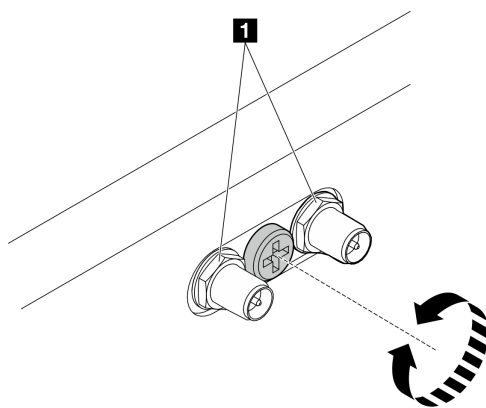
图 310. 缩短 SMA 接口
