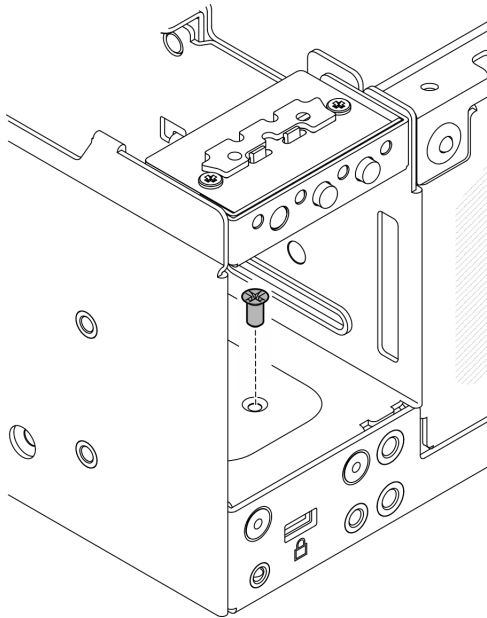
图 172. 拧紧螺钉
