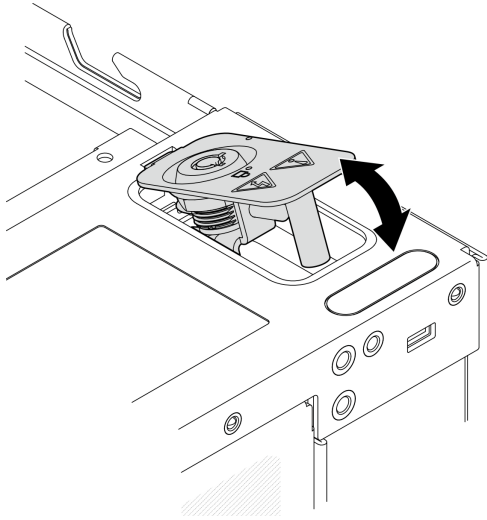
图 171. 安装系统安全钥匙锁
