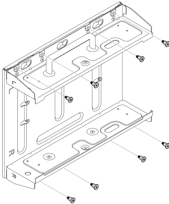
图 27. 卸下节点支架
