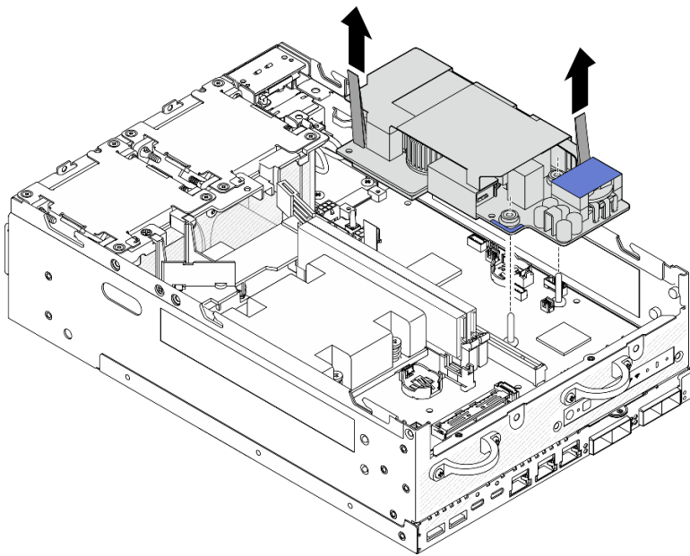
图 136. 卸下内部电源模块单元
