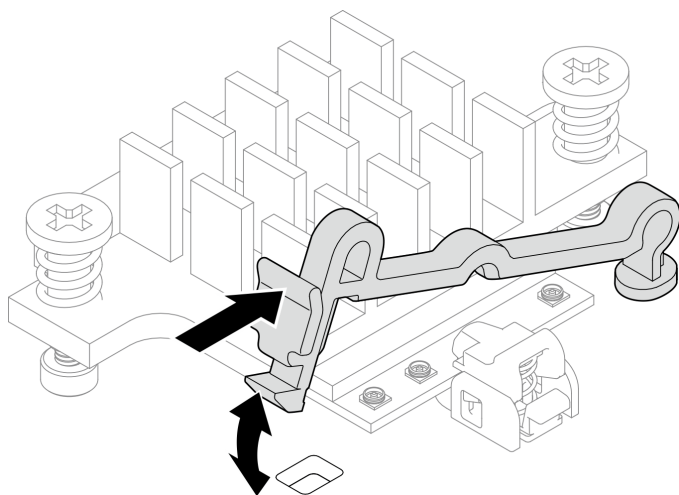
图 316. 插入线缆固定扣
