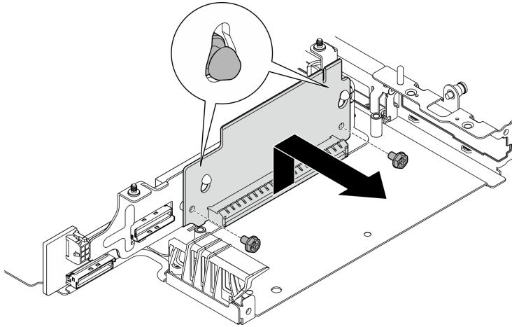
图 240. 卸下转接卡
