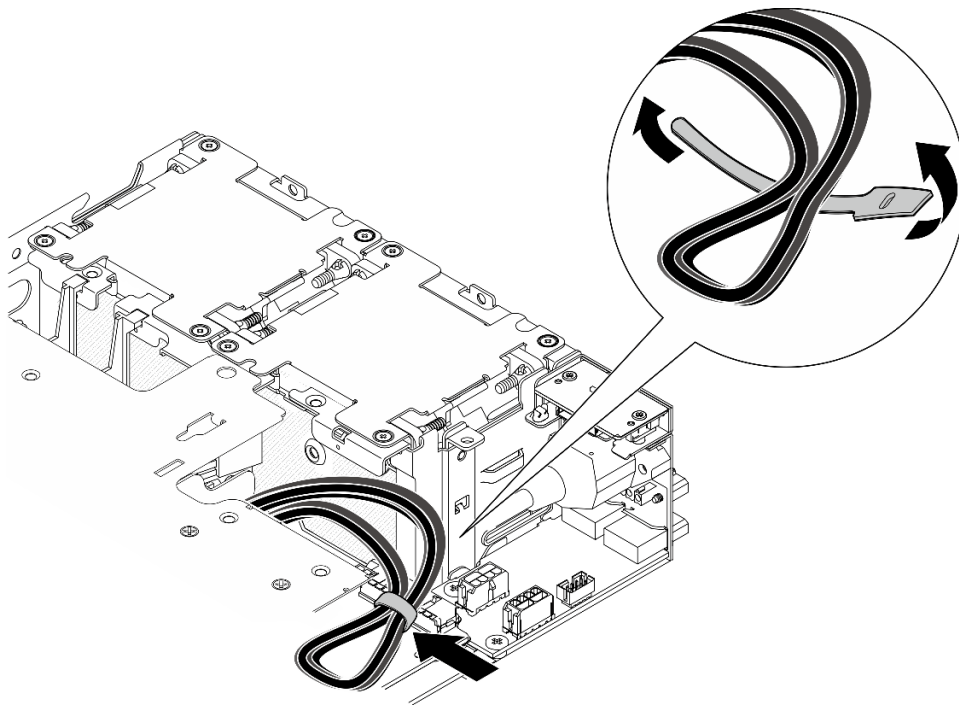
图 262. 转接卡组合件的线缆布放
