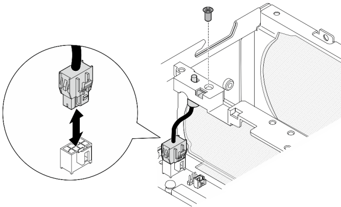
图 125. 安装风扇方向开关
