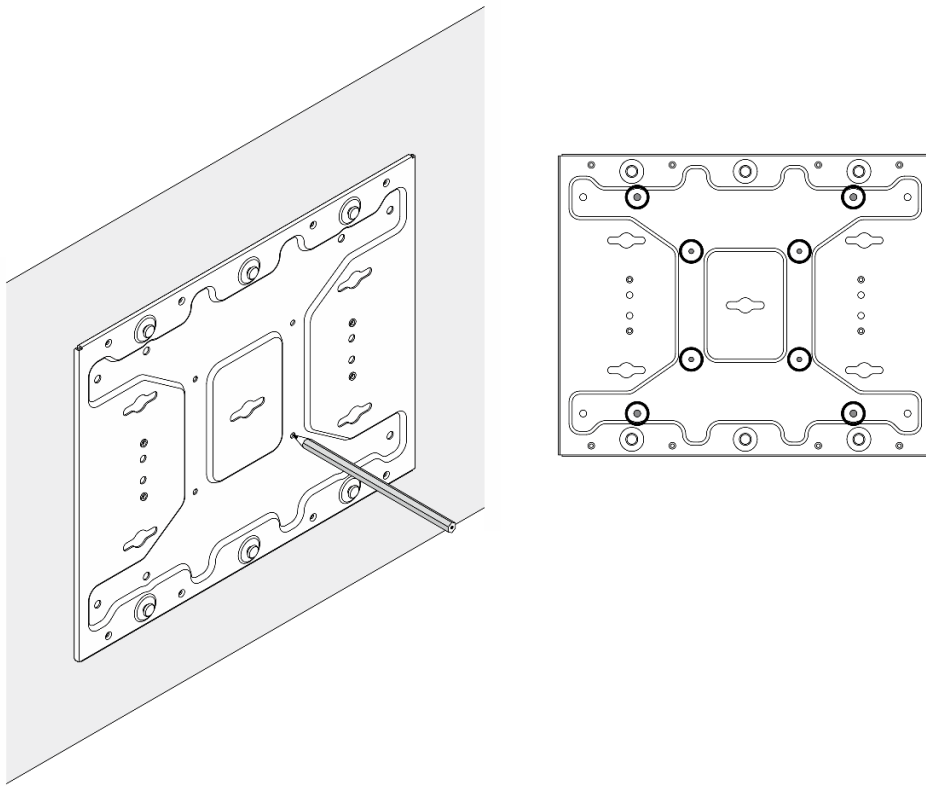
图 43. 螺钉孔的位置
