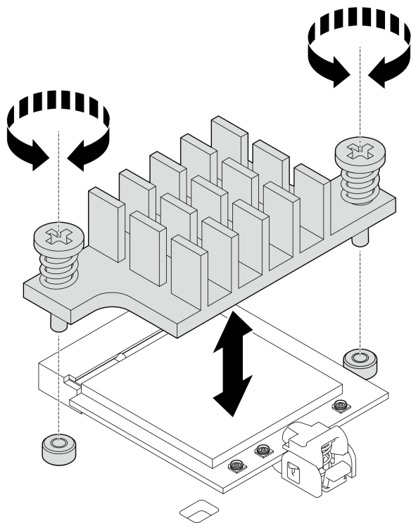
图 289. 安装 WLAN/蓝牙模块散热器
