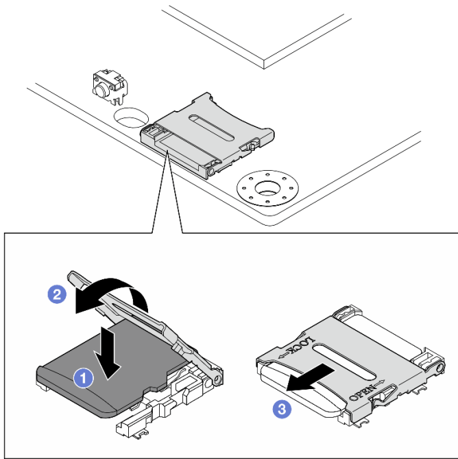
图 183. 安装 MicroSD 卡
