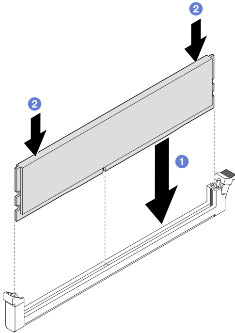
图 181. 安装内存条
