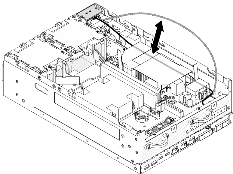
图 141. 放置信号线缆
