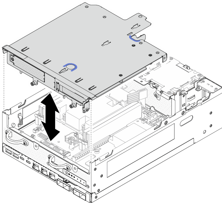
图 263. 下放转接卡组合件
