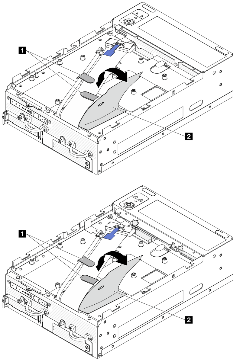
图 159. I/O 板线缆布放
