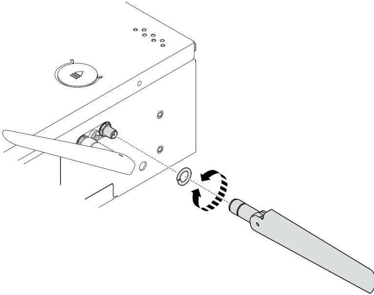
图 338. 安装 WLAN 天线
