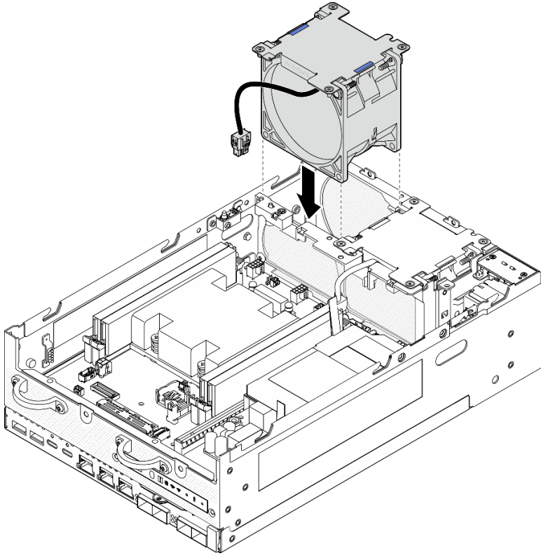
图 128. 安装风扇模块
