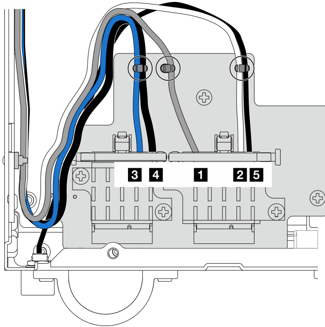
图 330. 无线适配器线缆布放
