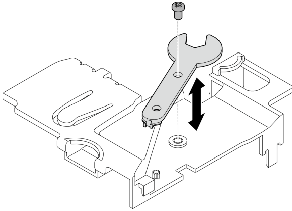
图 335. 存放扳手
