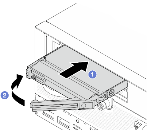
图 79. 安装 7 毫米硬盘
