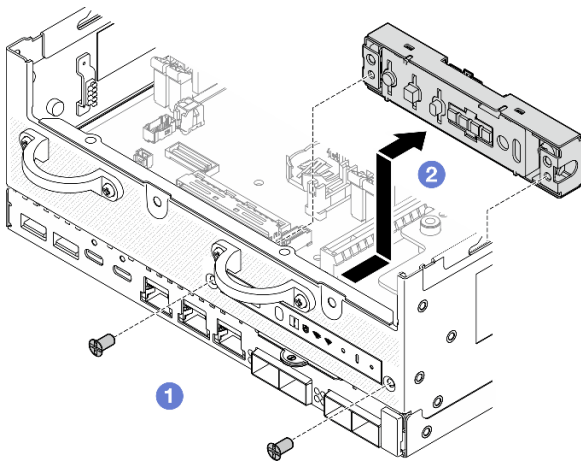
图 130. 卸下正面操作员面板
