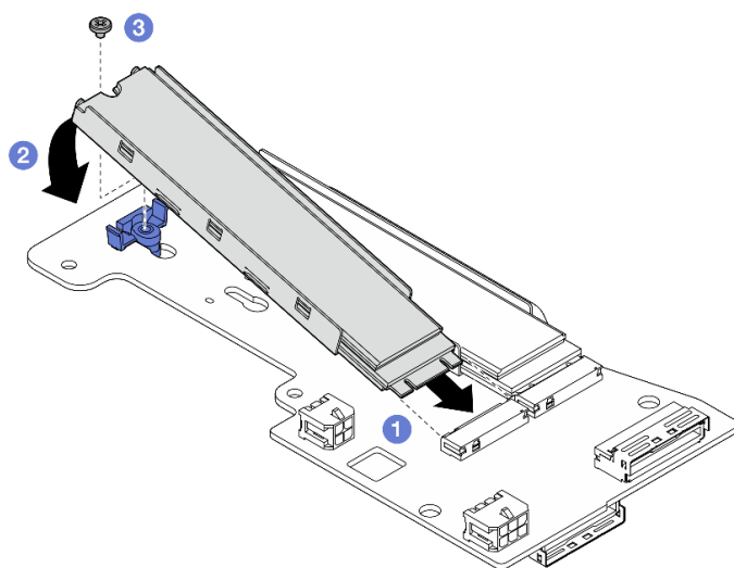
图 116. 安装 M.2 硬盘
