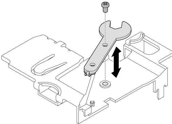
图 101. 存放扳手
