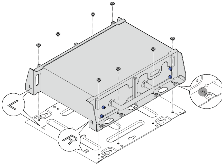
图 42. 安装底板
