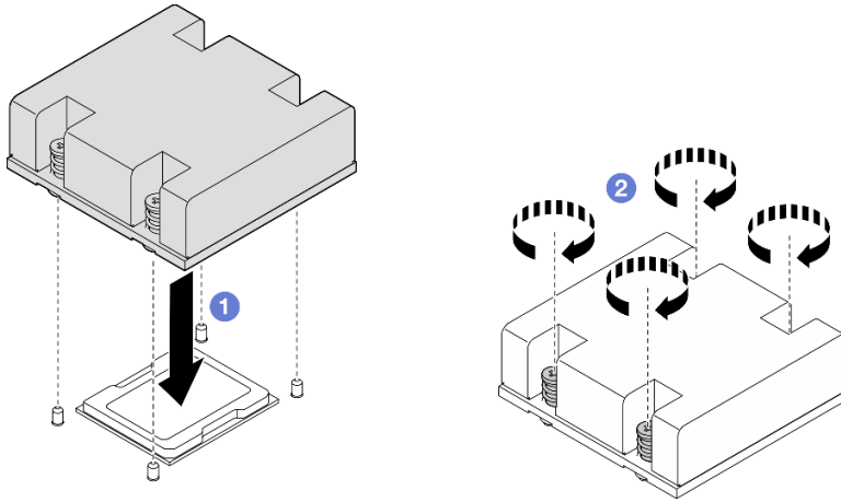
图 219. 安装处理器散热器
