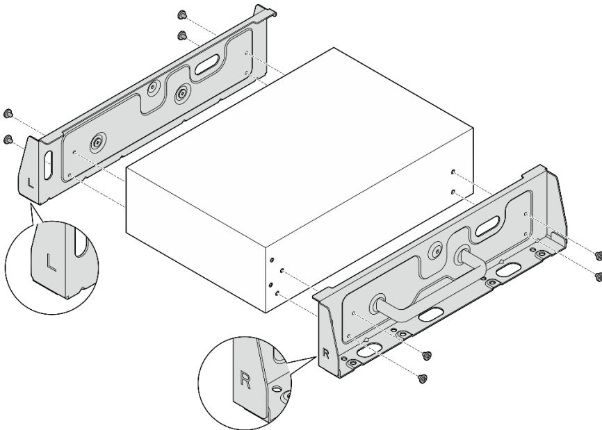
图 32. 松开螺钉以卸下侧面支架
