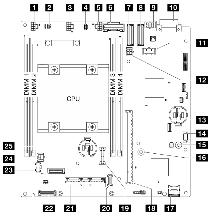
图 346. 主板接口
