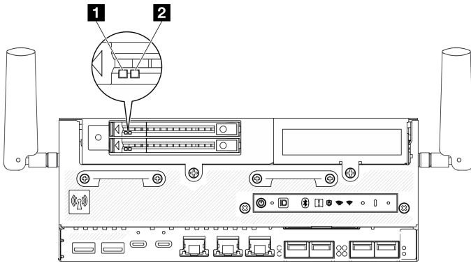
图 347. 硬盘 LED
