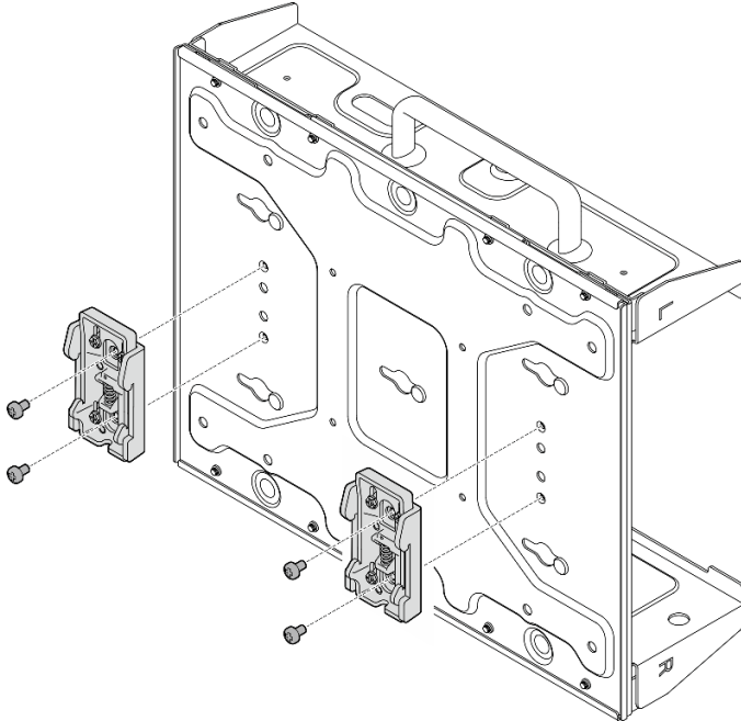
图 63. 安装 DIN 导轨夹
