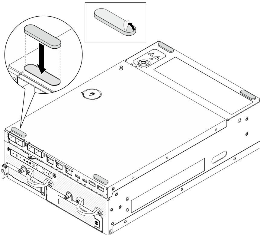
图 271. 安装橡胶支脚
