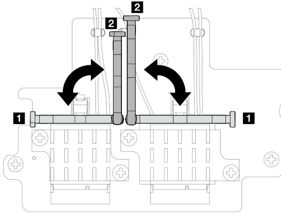
图 302. 转动线缆固定扣
