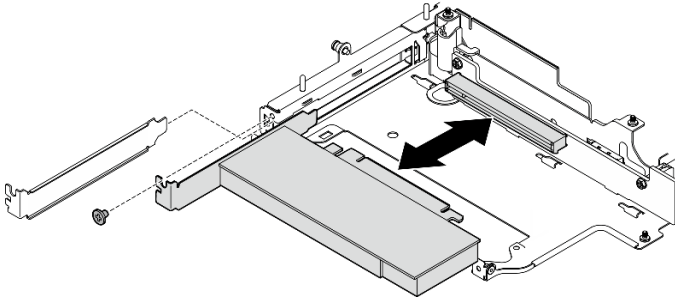
图 234. 卸下 PCIe 适配器
