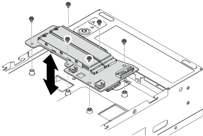
图 113. 卸下底部 M.2 有线适配器
