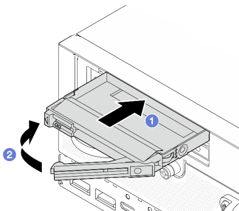
图 80. 安装硬盘填充件
