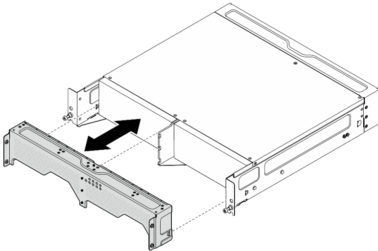
图 70. 安装装运支架
