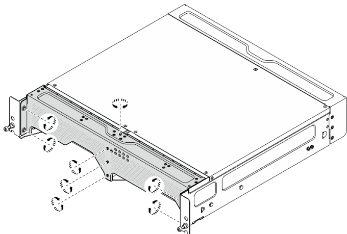
图 2. 拧松螺钉
