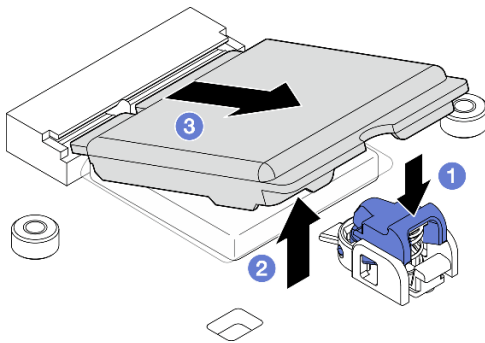
图 285. 卸下保护盖
