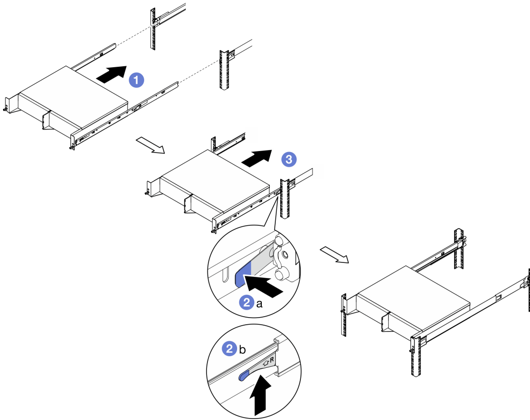
图 17. 将机柜安装到机架中
