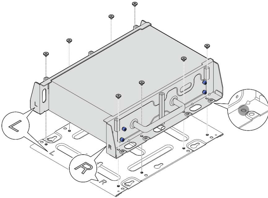
图 31. 卸下底板
