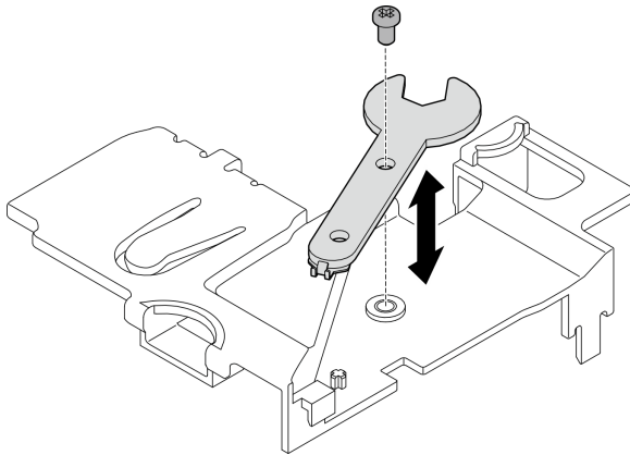
图 322. 取下扳手
