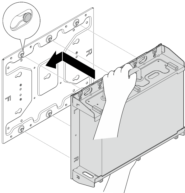
图 47. 安装节点支架
