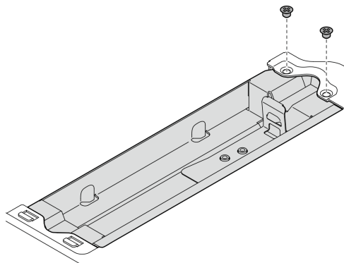
图 258. 安装 位置跟踪模块仓
