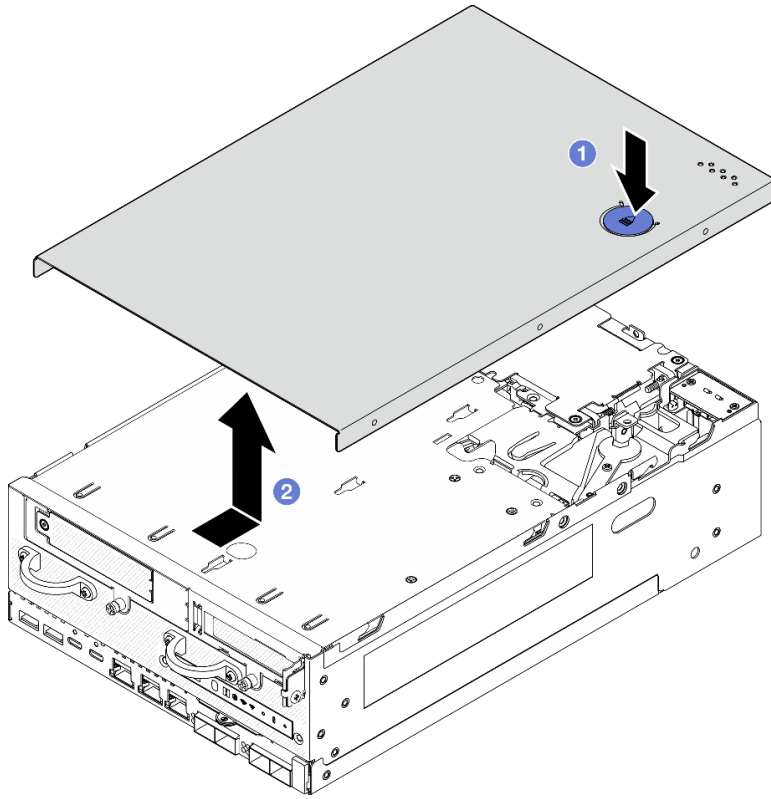
图 185. 卸下顶盖
