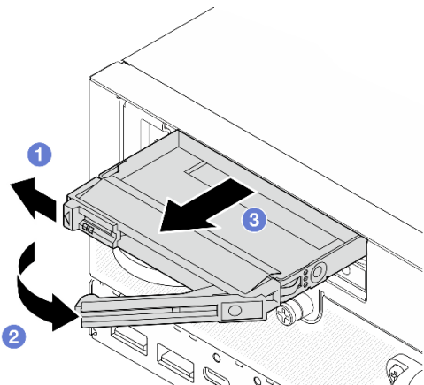
图 78. 卸下硬盘填充件
