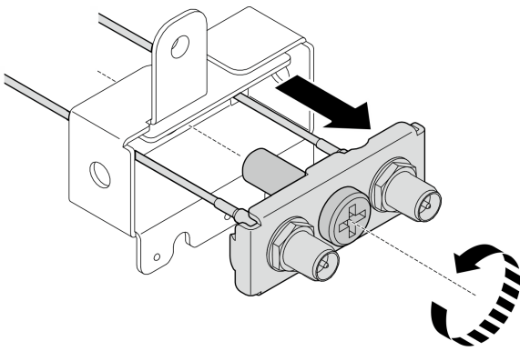
图 318. 卸下支架
