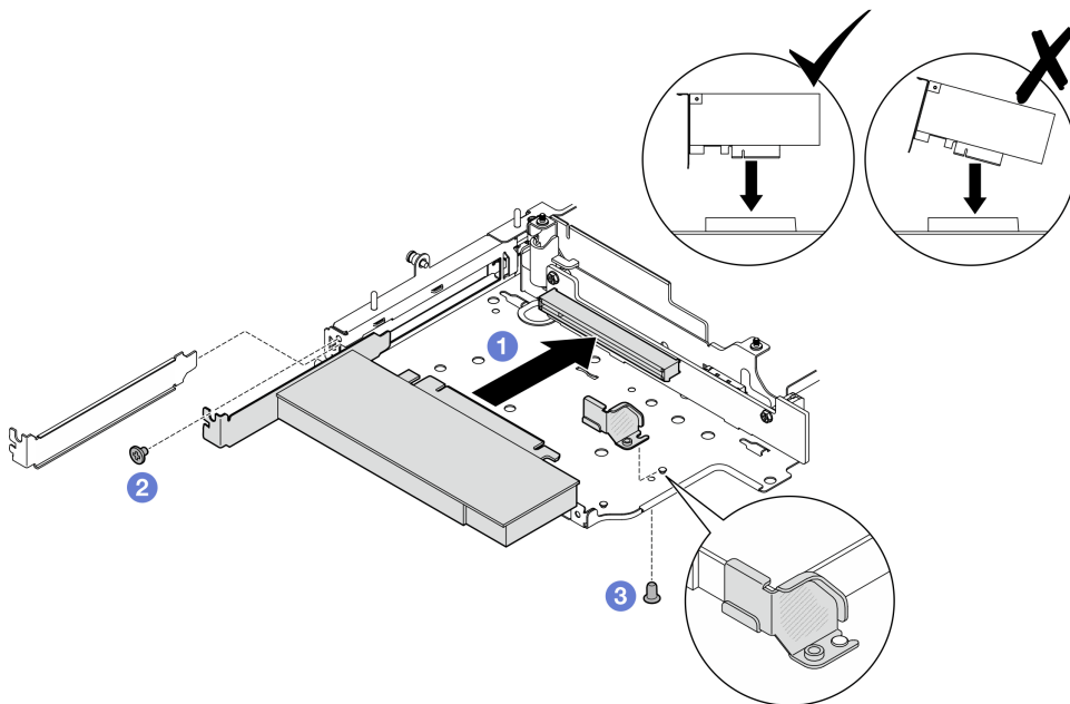
图 251. 安装 PCIe 适配器
