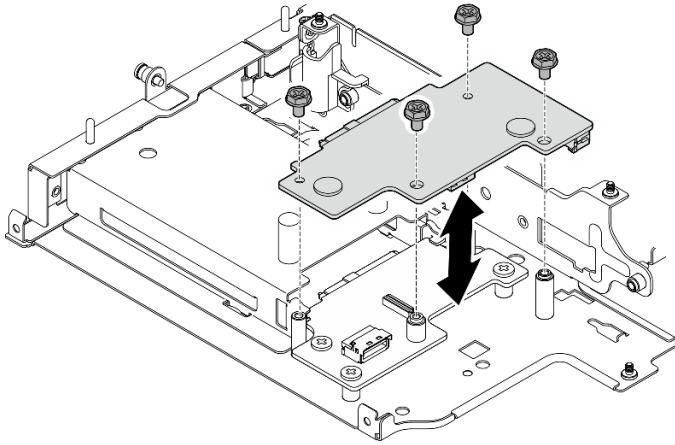
图 229. 卸下背板 2
