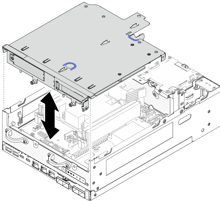
图 223. 提起转接卡组合件
