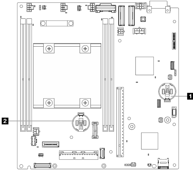
图 117. 主板上的 CMOS 电池位置
