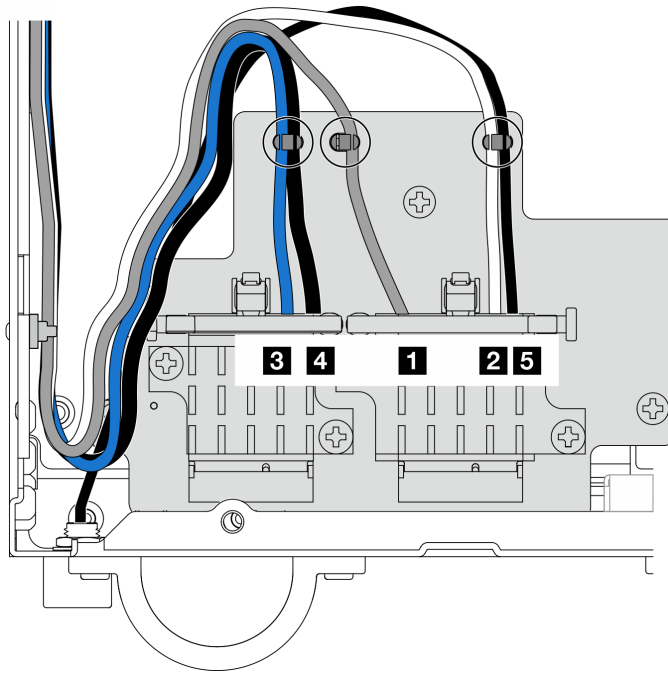
图 334. 无线适配器线缆布放
