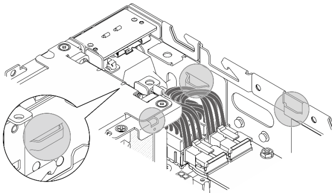
图 213. PMB 导风罩的插槽
