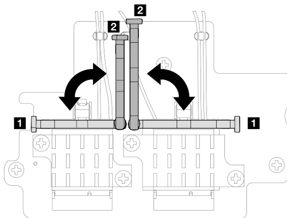
图 329. 转动线缆固定扣
