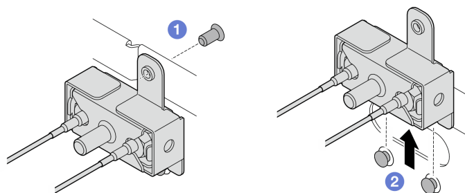
图 306. 卸下 SMA 组合件
