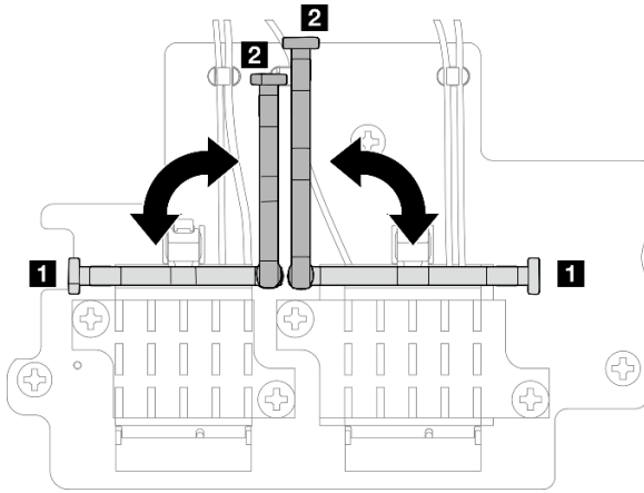
图 313. 转动线缆固定扣
