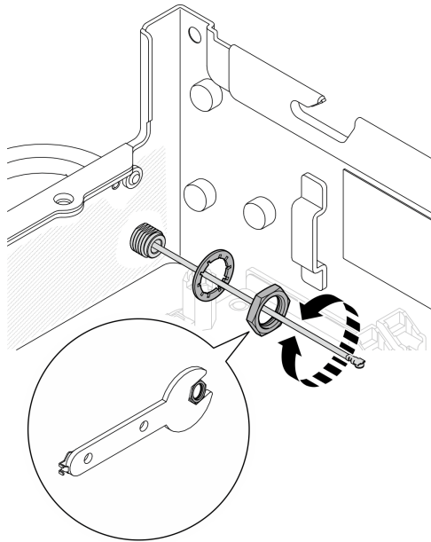
图 99. 卸下蓝牙天线
