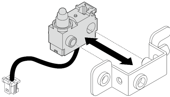
图 151. 将入侵感应开关插入支架
