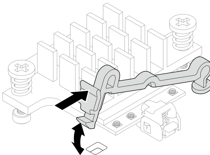
图 312. 提起线缆固定扣
