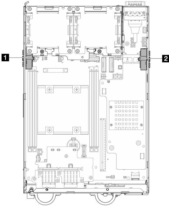
图 297. SMA 组合件位置
