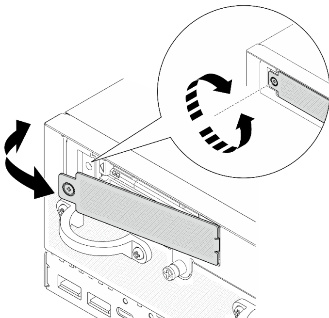
图 81. 安装挡板
