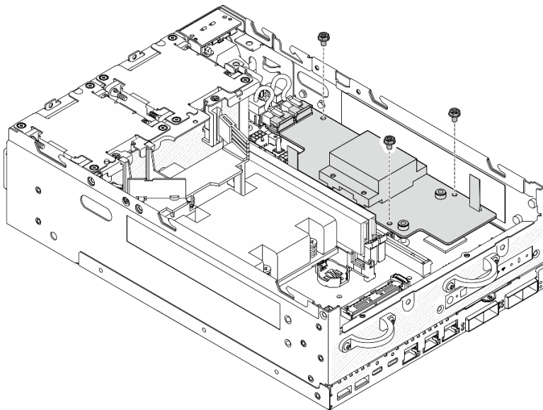
图 209. 拧松螺钉
