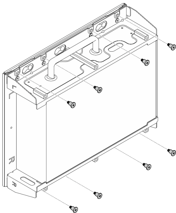
图 48. 安装节点支架
