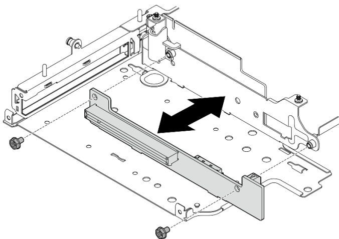
图 254. 安装转接卡
