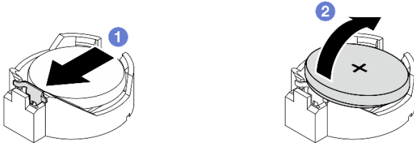
图 119. 卸下 CMOS 电池
