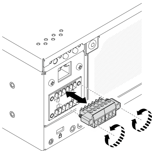
图 205. 拔下接头
