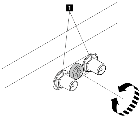
图 30. 缩短 SMA 接口
