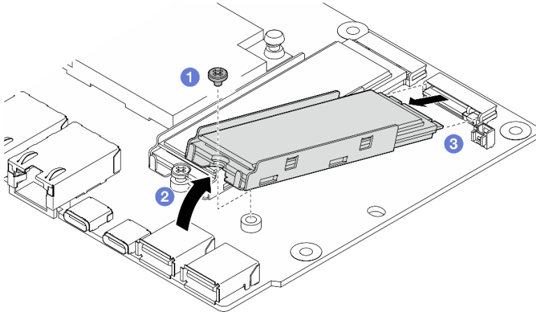
图 154. 卸下 M.2 硬盘
