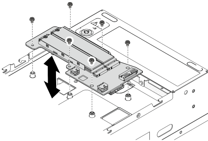
图 115. 安装底部 M.2 有线适配器
