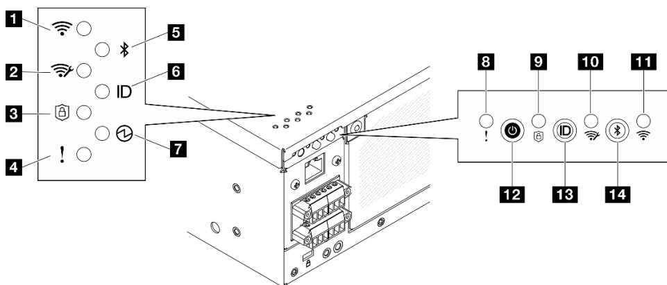
图 350. 背面操作员面板 LED
