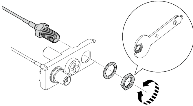
图 325. 将线缆紧固在支架上
