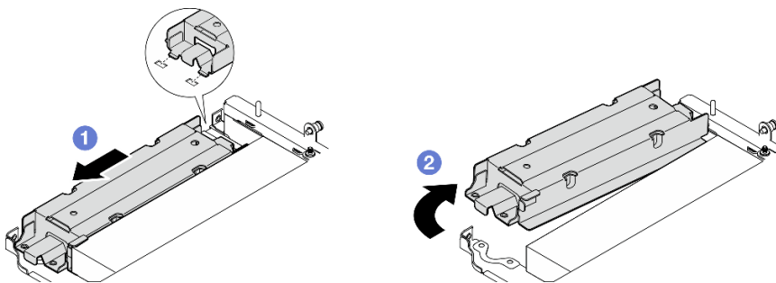
图 233. 卸下位置跟踪模块仓
