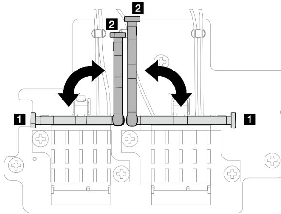
图 108. 转动线缆固定扣
