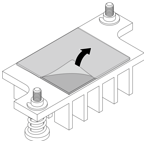
图 288. 撕下导热垫上的薄膜
