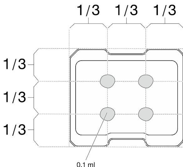
图 218. 导热油脂的正确形状
