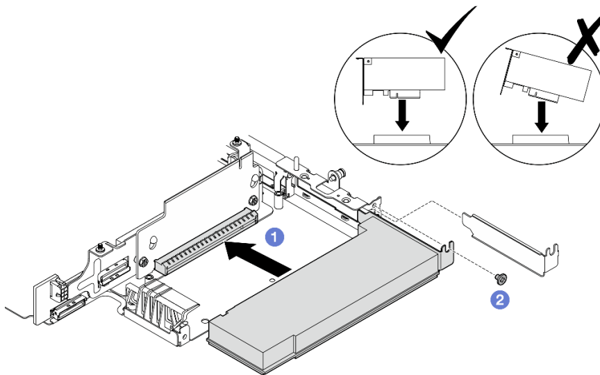
图 245. 安装 PCIe 适配器
