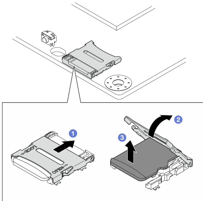
图 182. 卸下 MicroSD 卡
