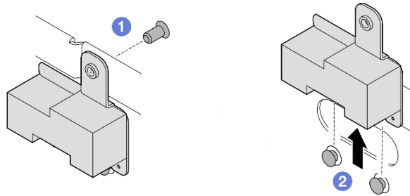
图 311. 卸下 SMA 填充件
