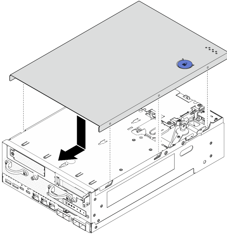
图 188. 安装顶盖
