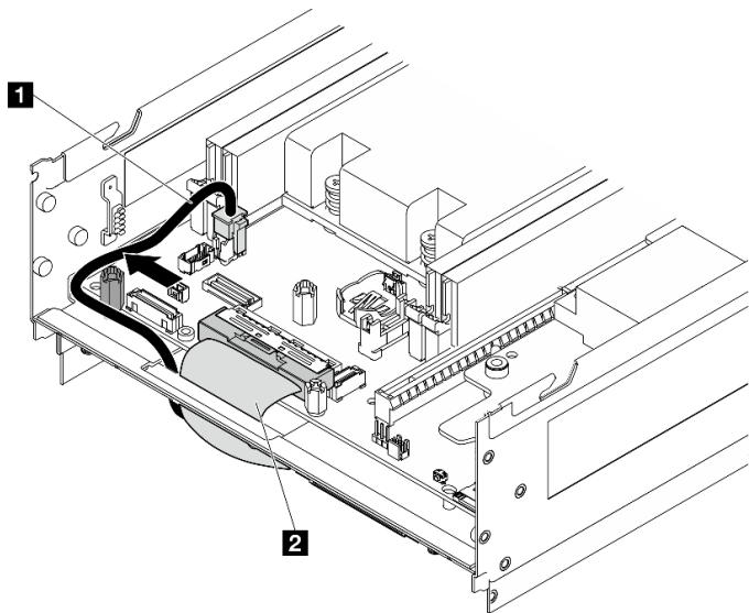
图 276. I/O 板线缆布放
