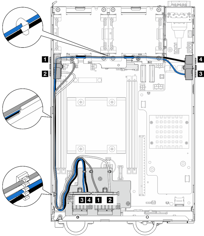
图 342. WLAN 天线线缆布放
