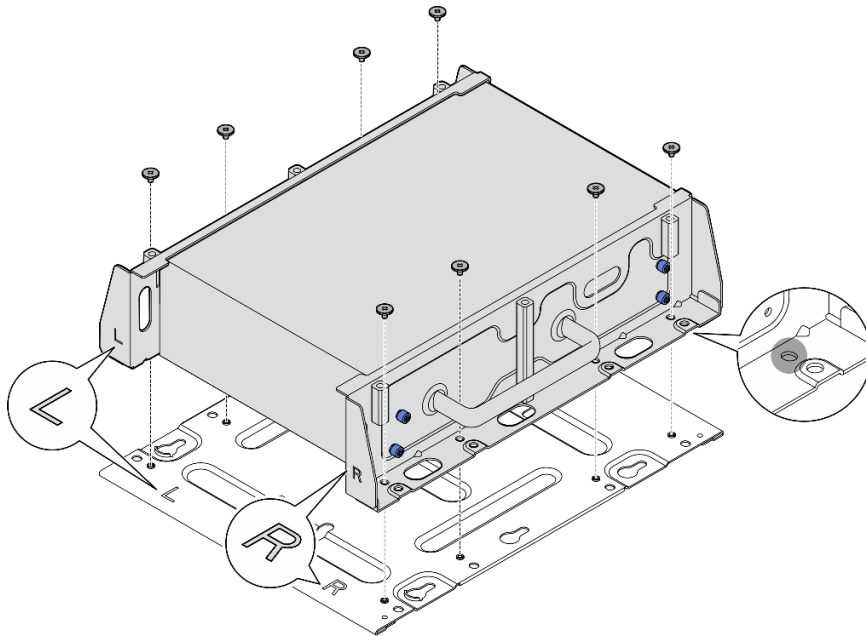
图 54. 卸下底板
