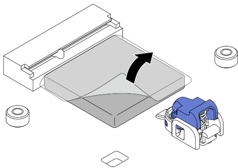
图 286. 撕下导热垫上的薄膜
