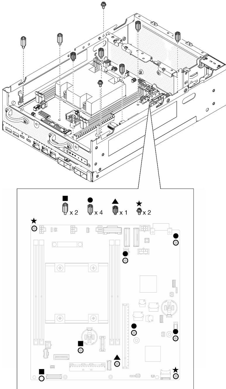
图 272. 主板上的螺钉和支脚
