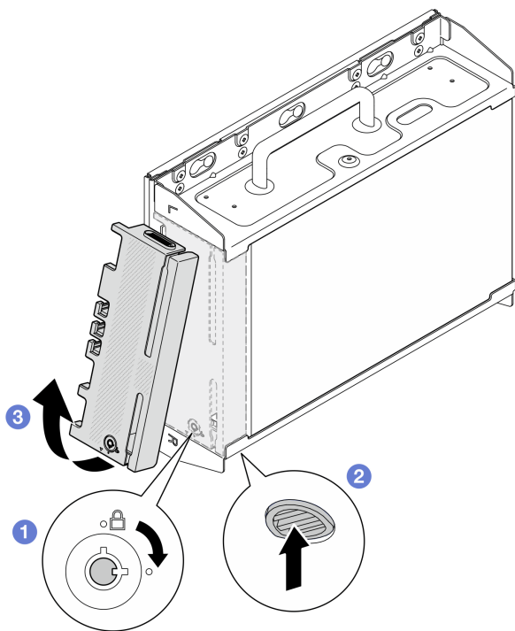
图 50. 卸下安全挡板
