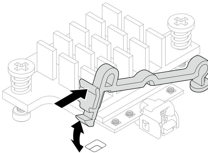
图 305. 插入线缆固定扣
