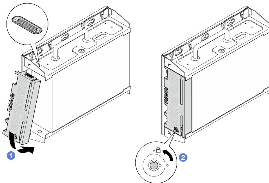
图 49. 安装安全挡板
