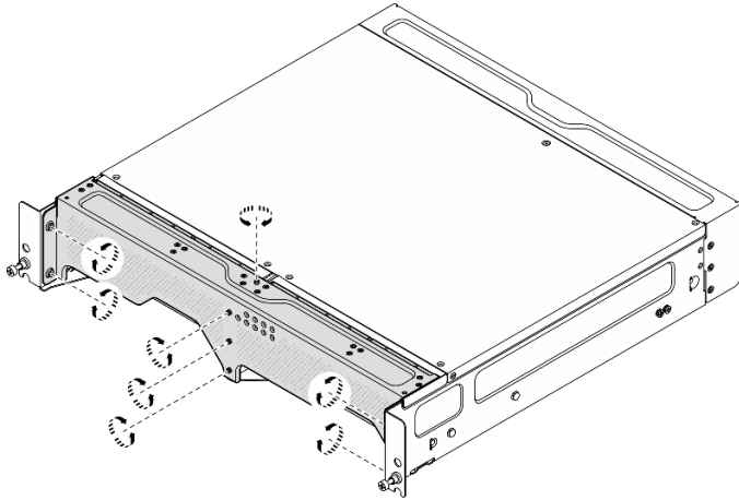
图 71. 拧紧螺钉
