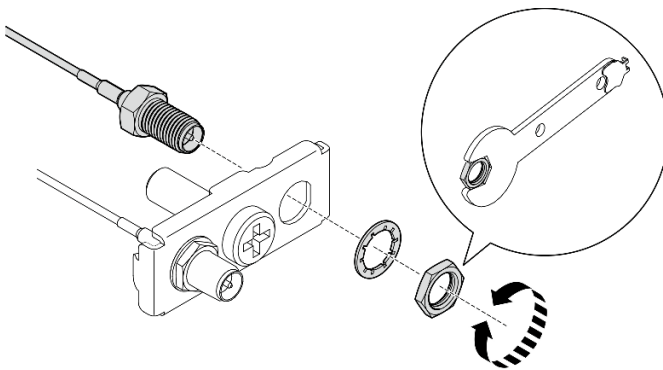
图 319. 从支架上松开线缆
