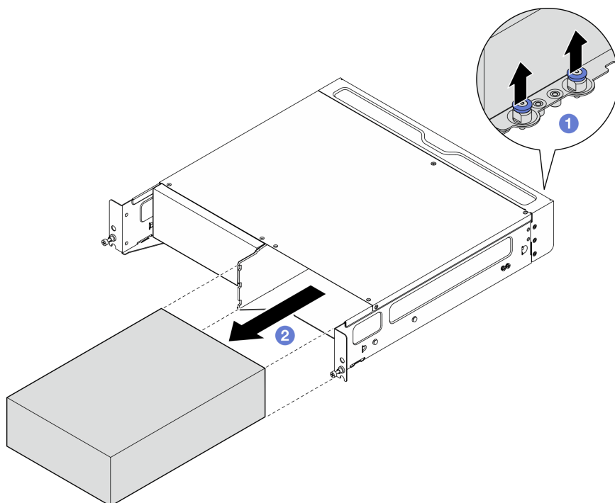
图 4. 卸下节点
