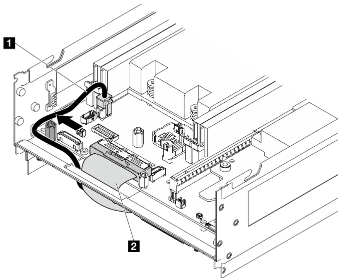
图 157. I/O 板线缆布放
