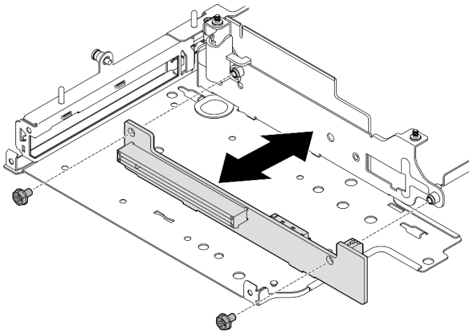
图 235. 卸下转接卡
