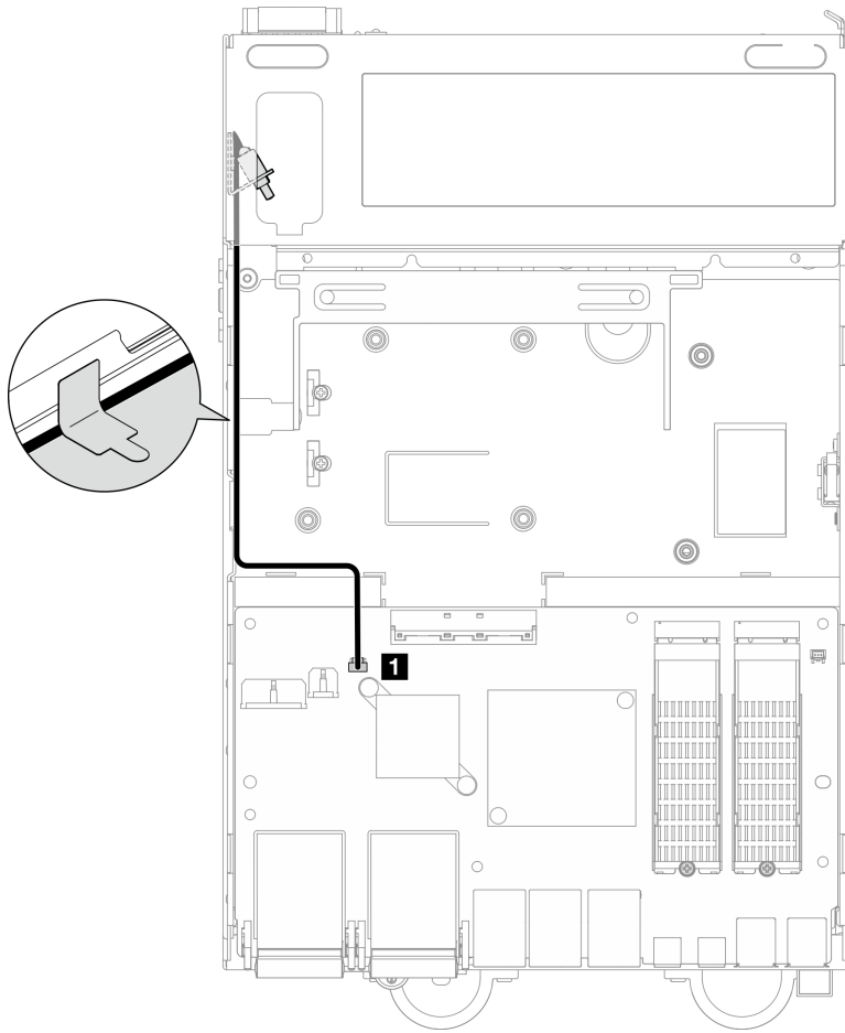
图 170. 锁定位置开关线缆布放
