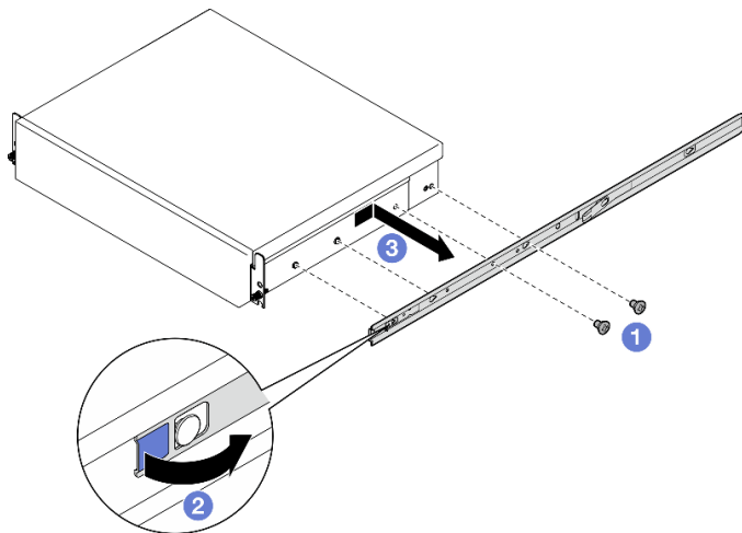
图 9. 卸下内侧导轨
