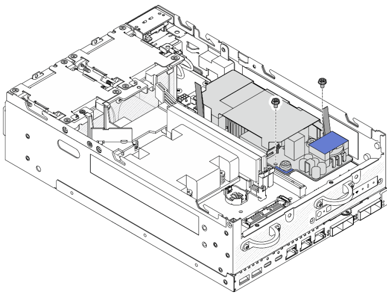
图 139. 拧紧螺钉
