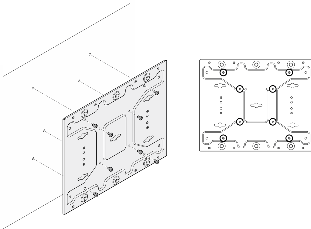
图 44. 安装壁挂板
