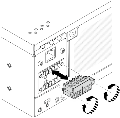
图 339. 安装接头
