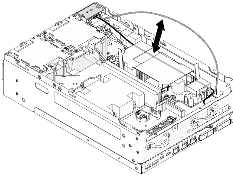
图 132. 放置信号线缆
