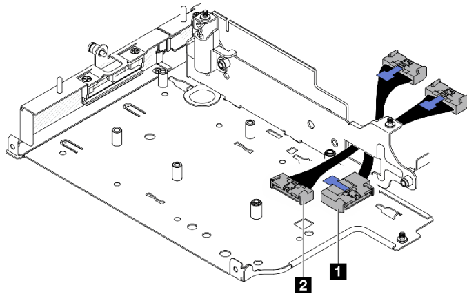
图 247. M.2 有线适配器信号线缆
