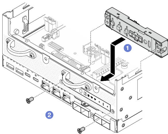
图 131. 安装正面操作员面板
