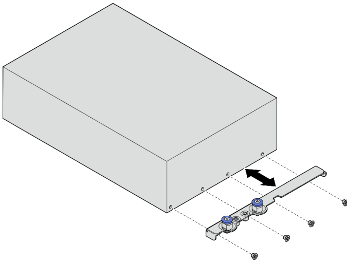
图 6. 卸下机柜支架
