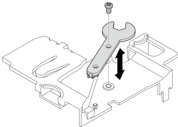
图 92. 取下扳手
