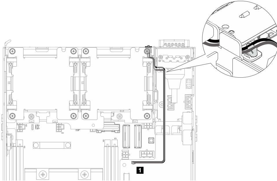
图 196. 连接到直流电源模块板（直流 PMB）的 PMB 状态 LED 线缆
