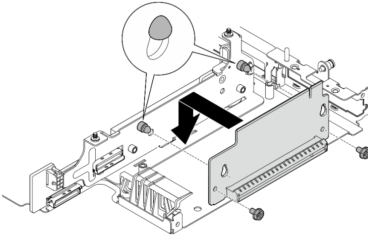
图 244. 安装转接卡
