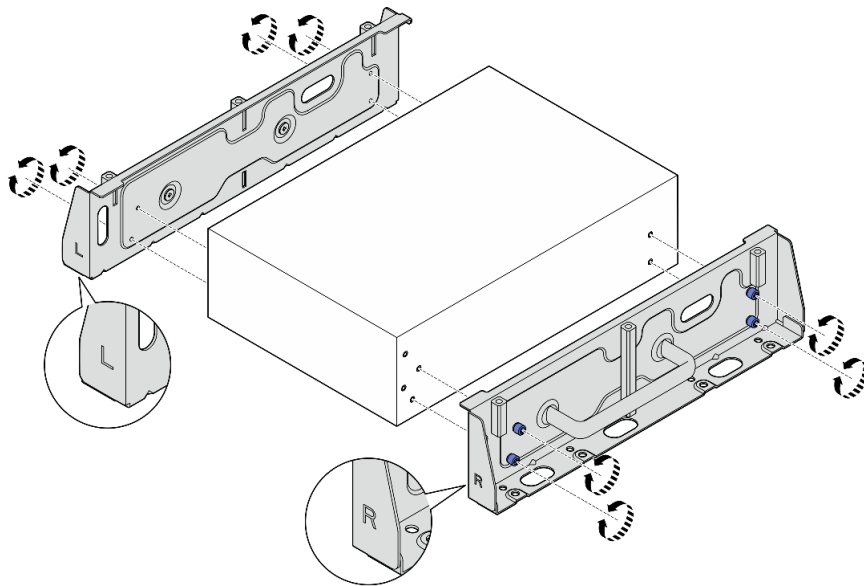
图 56. 松开指旋螺钉以卸下侧面支架
