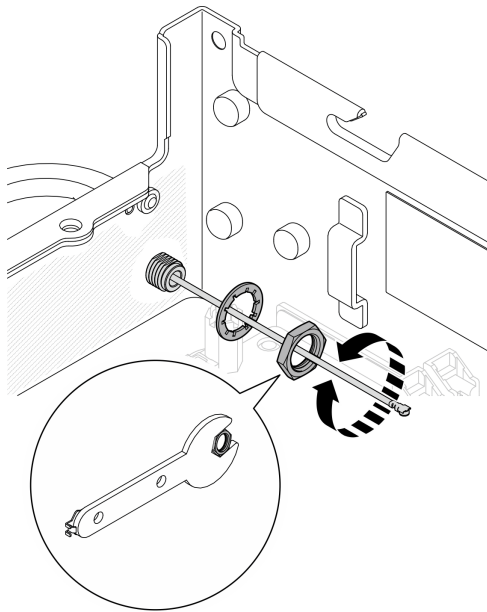
图 104. 安装蓝牙天线
