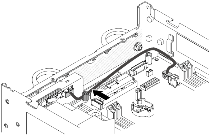
图 341. 正面操作员面板线缆布放
