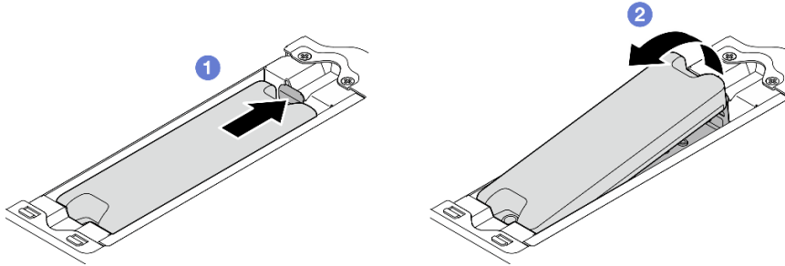
图 231. 卸下位置跟踪模块
