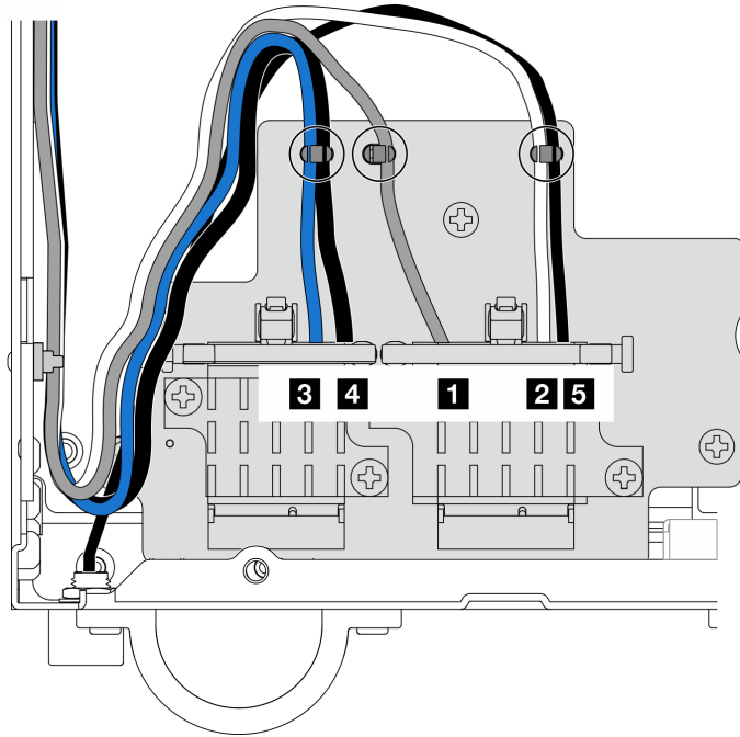
图 290. 无线适配器线缆布放
