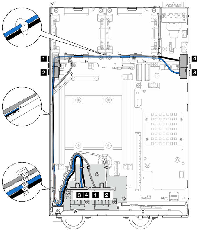
图 327. SMA 组合件的线缆布放
