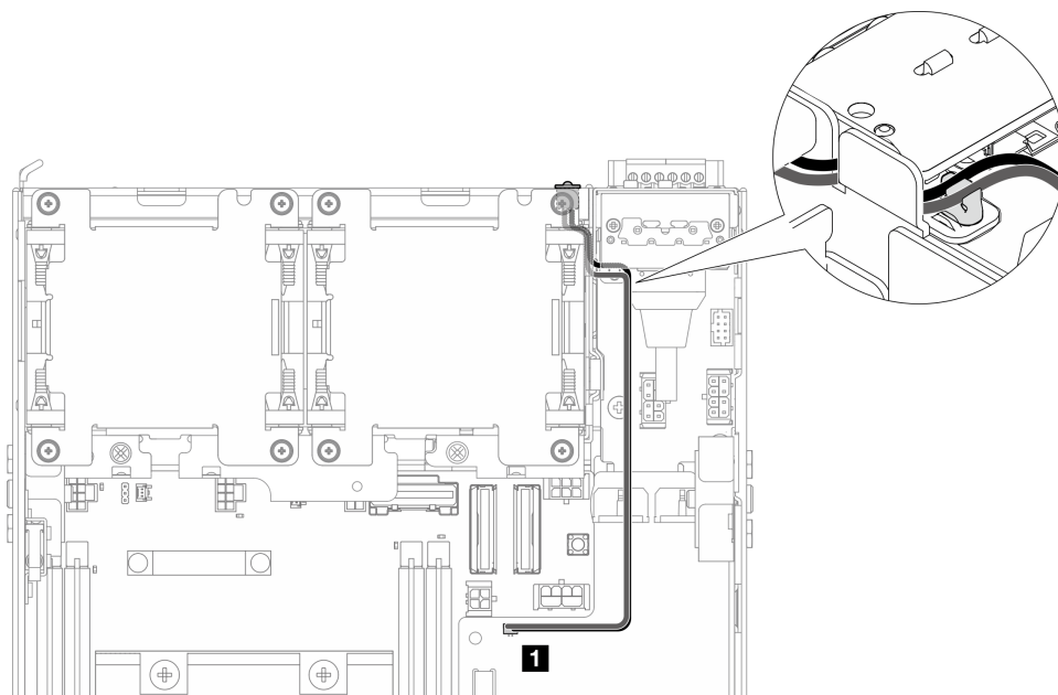
图 200. 连接到直流电源模块板（直流 PMB）的 PMB 状态 LED 线缆
