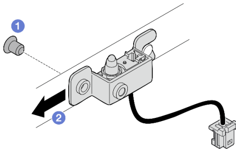
图 143. 卸下带线缆的入侵感应开关
