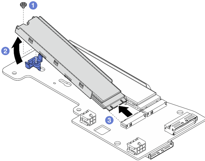
图 226. 卸下 M.2 硬盘
