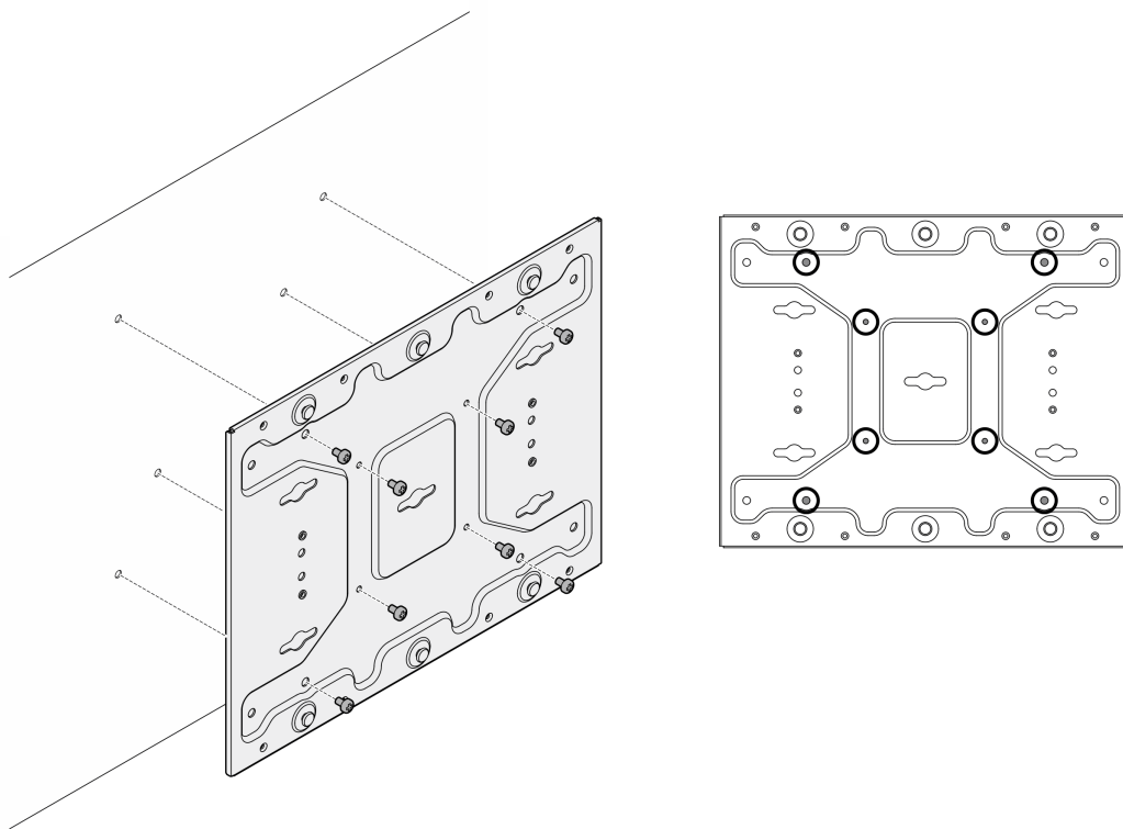
图 29. 卸下壁挂板
