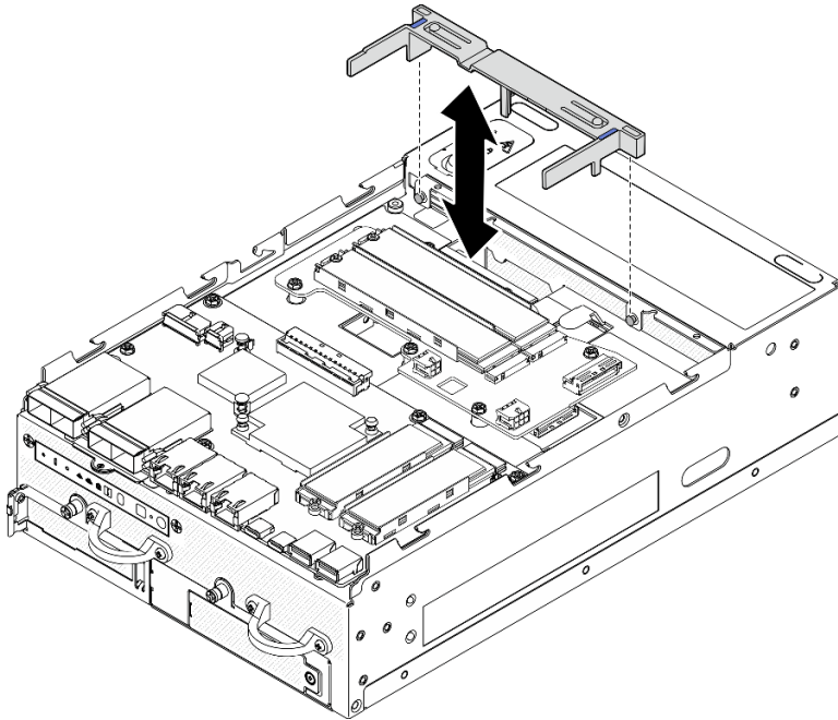
图 83. 安装导风罩
