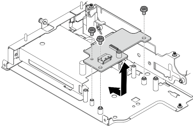
图 230. 卸下背板 1
