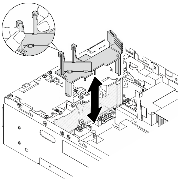
图 89. 安装导风罩
