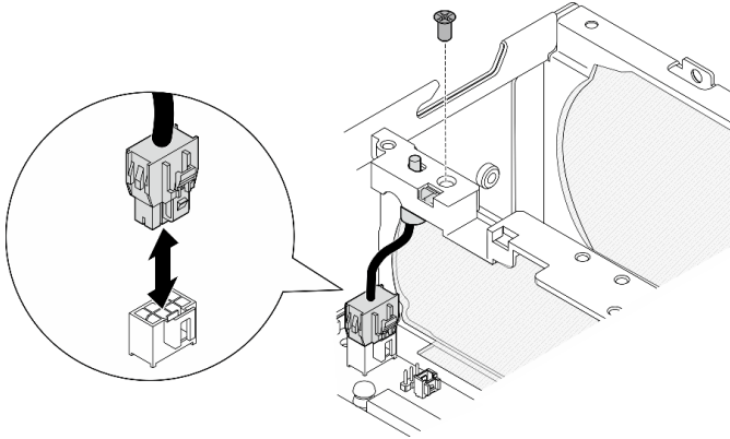
图 122. 卸下风扇方向开关
