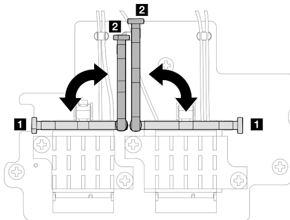
图 97. 转动线缆固定扣
