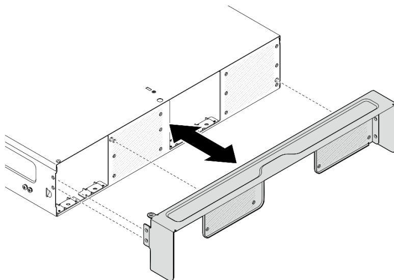
图 12. 安装装运支架
