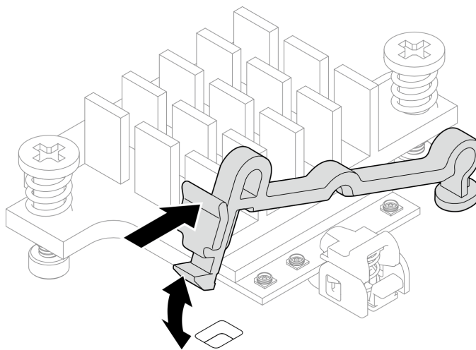
图 278. 提起线缆固定扣
