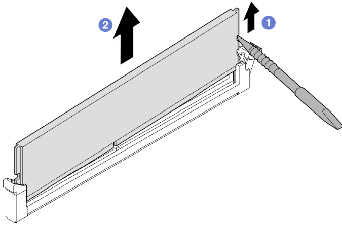
图 178. 卸下内存条
