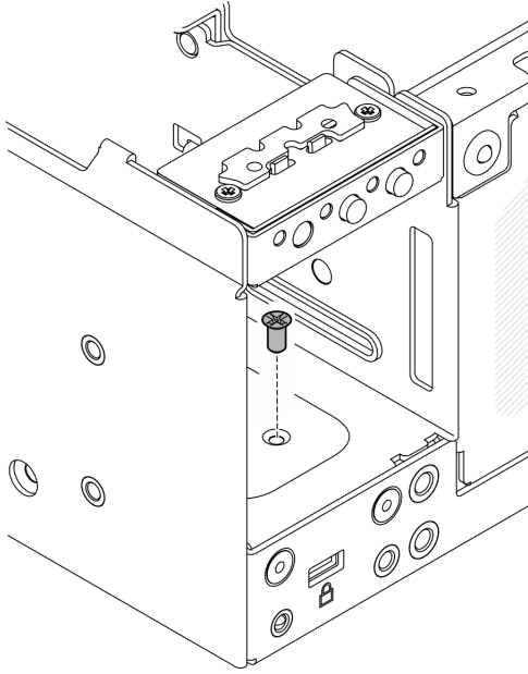
图 165. 拧松螺钉
