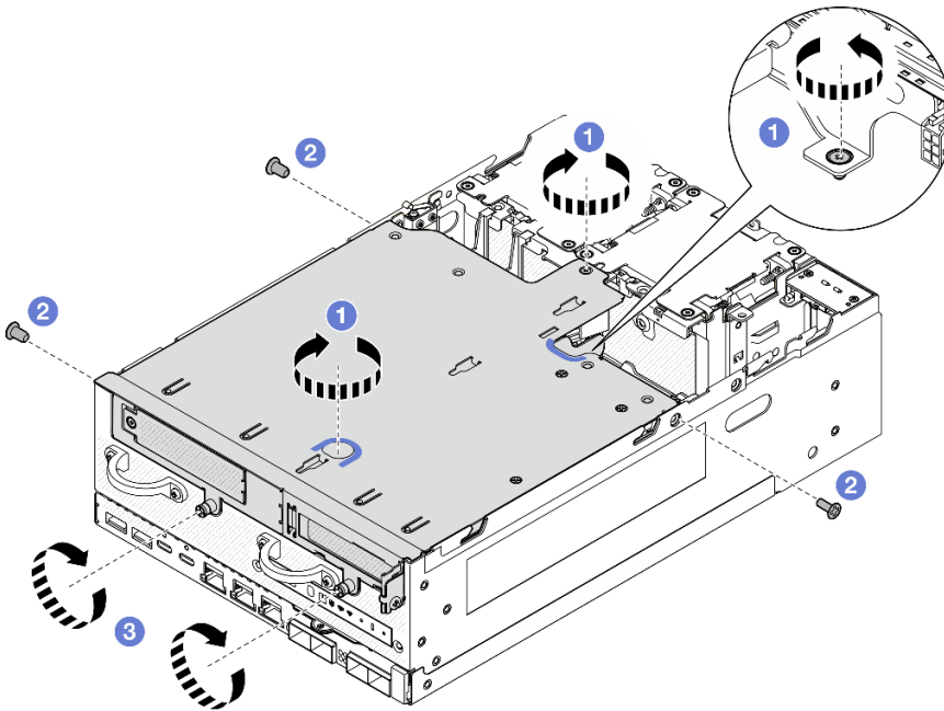
图 265. 固定转接卡组合件
