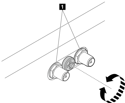
图 337. 伸出 SMA 接口
