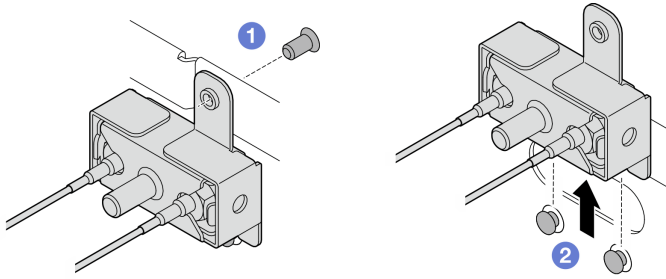
图 317. 卸下 SMA 组合件
