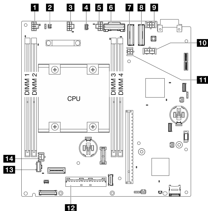
图 340. 主板接口
