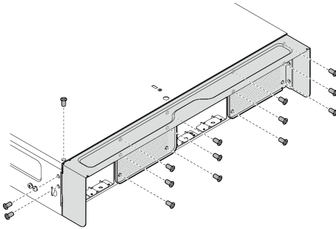
图 13. 拧紧螺钉
