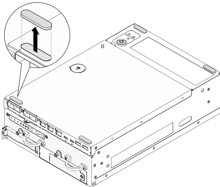
图 270. 卸下橡胶支脚
