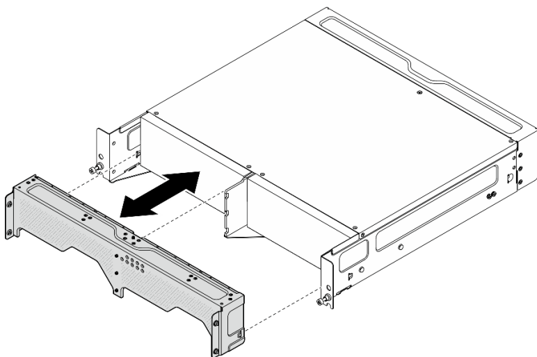
图 67. 卸下装运支架
