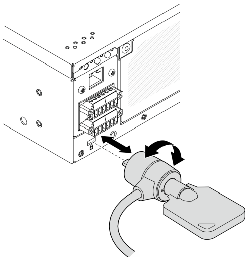
图 163. 卸下 Kensington 锁
