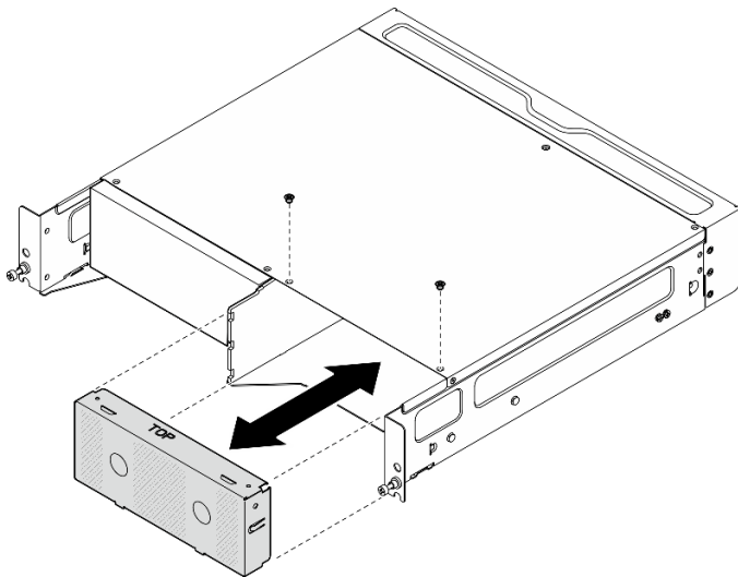
图 21. 卸下节点填充件
