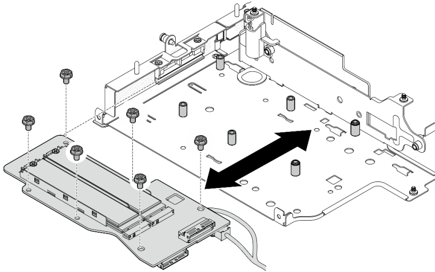
图 248. 安装 M.2 适配器
