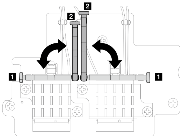
图 315. 转动线缆固定扣
