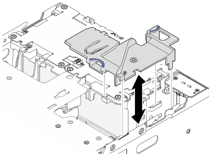
图 85. 安装导风罩
