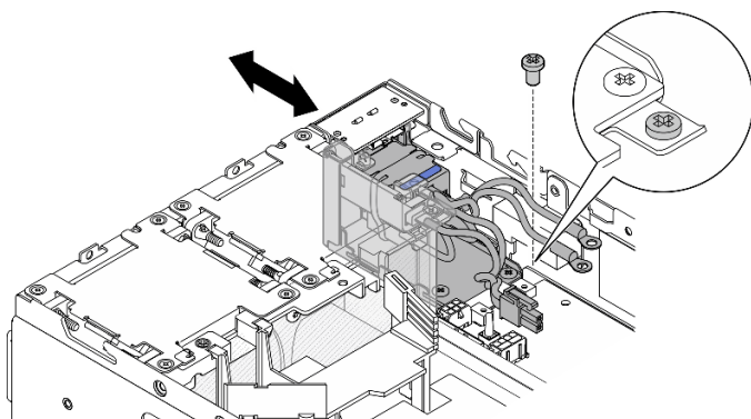
图 203. 卸下交流 PIB 模块
