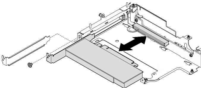
图 255. 安装 PCIe 适配器
