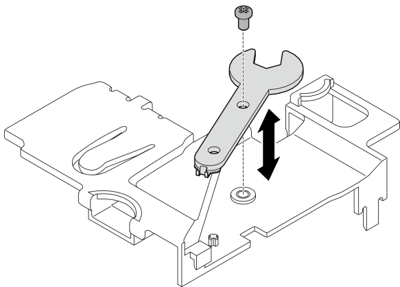
图 111. 存放扳手
