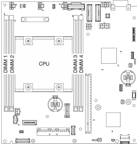
图 176. 内存条和处理器布局
