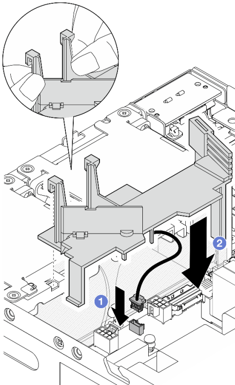
图 91. 安装导风罩
