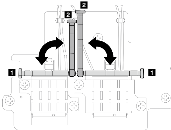
图 332. 转动线缆固定扣
