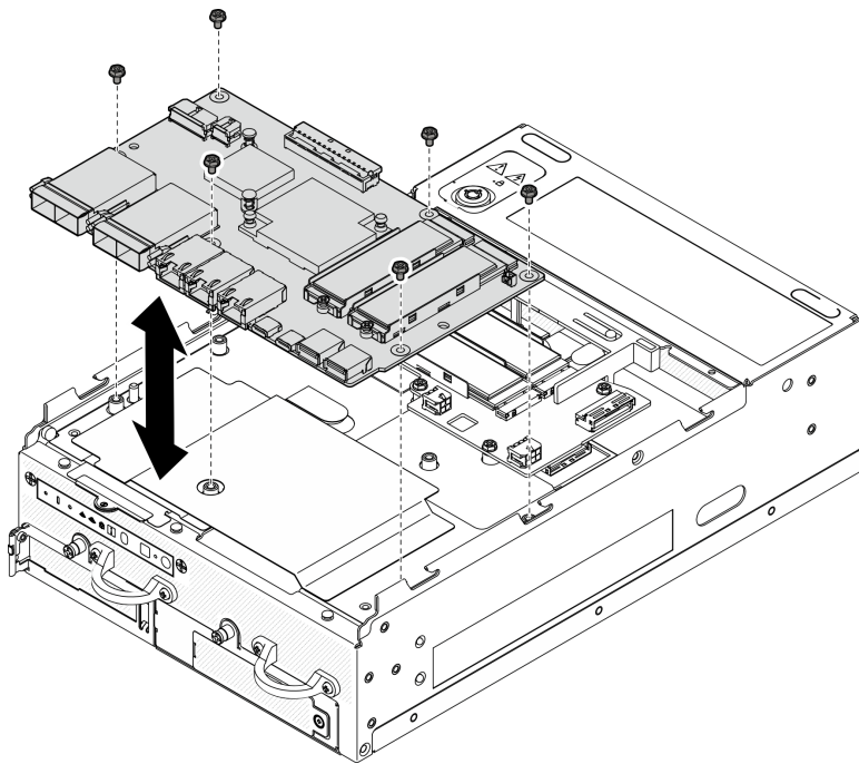
图 155. 卸下 I/O 模块板
