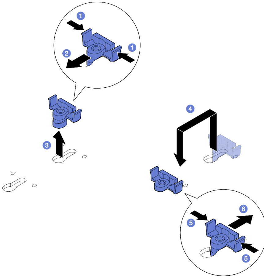
图 114. 调整 M.2 固定器
