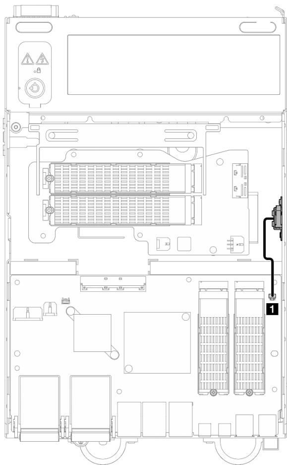
图 153. 底部入侵感应开关线缆布放
