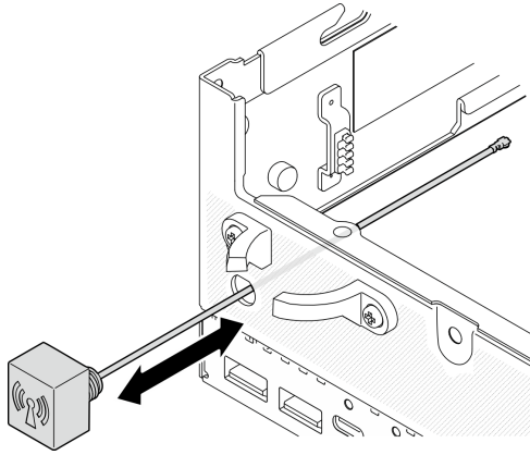
图 103. 安装蓝牙天线
