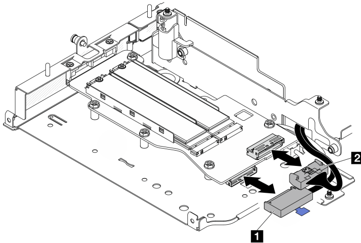
图 224. 拔下信号线缆
