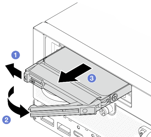
图 77. 卸下 7 毫米硬盘
