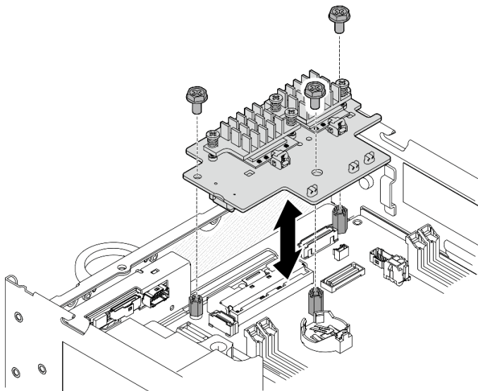
图 93. 提起无线适配器
