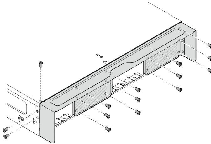
图 10. 拧松螺钉
