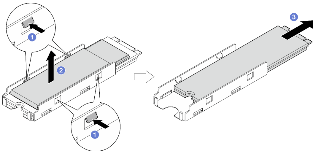
图 173. 卸下 M.2 散热器
