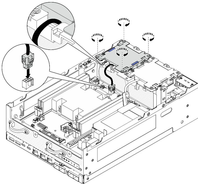
图 129. 安装风扇模块
