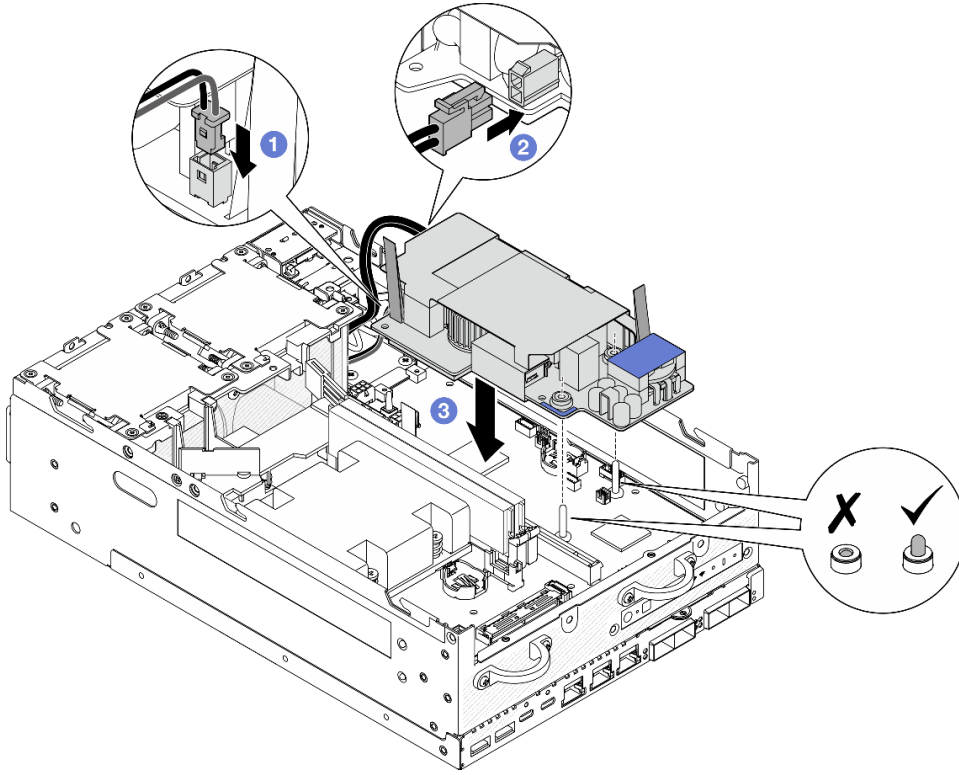
图 138. 安装内部电源模块单元
