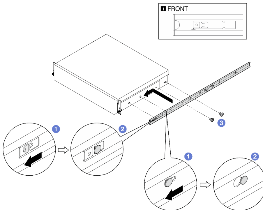
图 16. 安装内侧导轨
