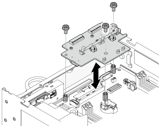
图 284. 安装无线适配器
