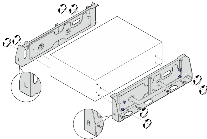
图 41. 用指旋螺钉安装侧面支架
