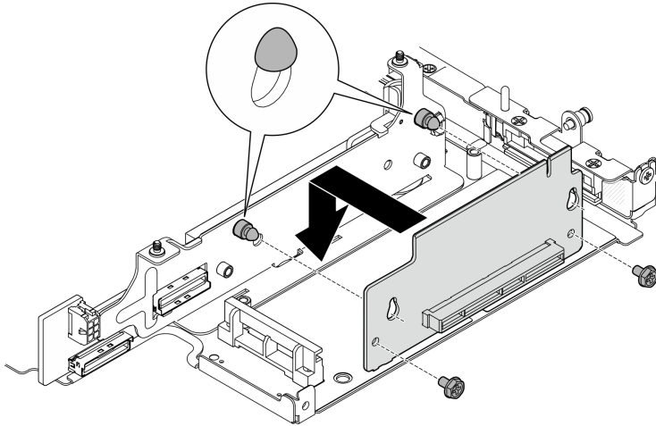
图 242. 安装转接卡
