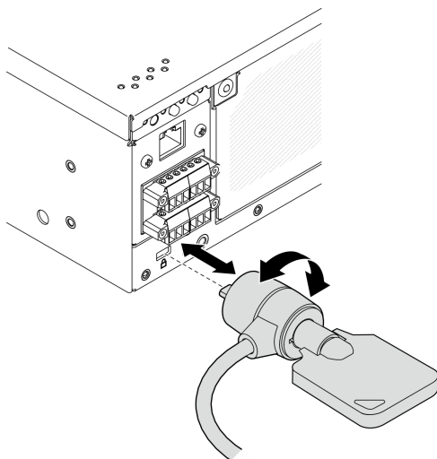
图 164. 安装 Kensington 锁
