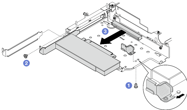
图 227. 卸下 PCIe 适配器
