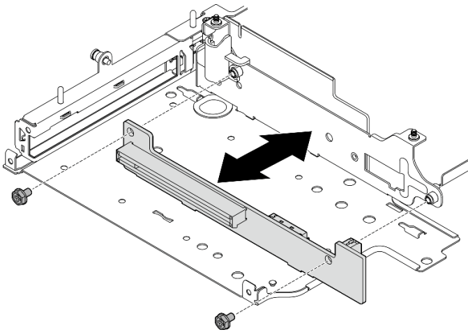
图 250. 安装转接卡
