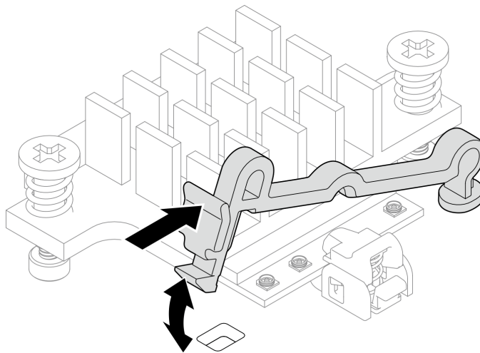
图 301. 提起线缆固定扣
