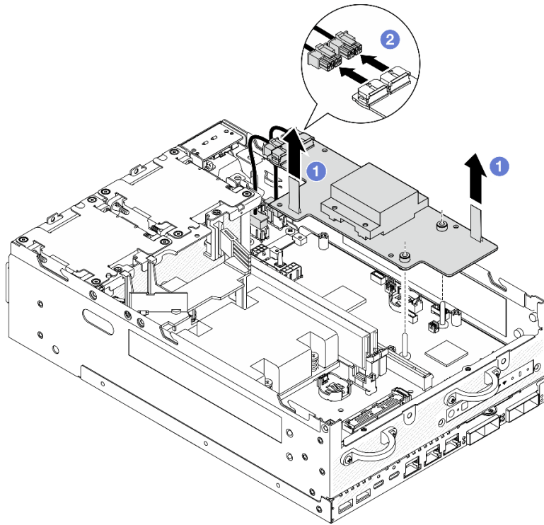
图 210. 卸下电源模块板
