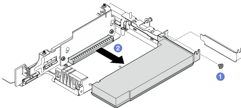
图 239. 卸下 PCIe 适配器
