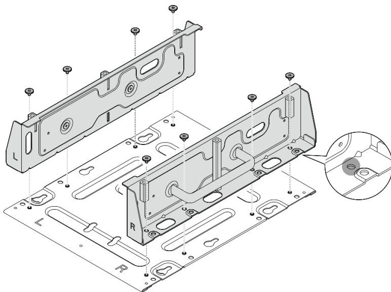
图 57. 组装节点套筒
