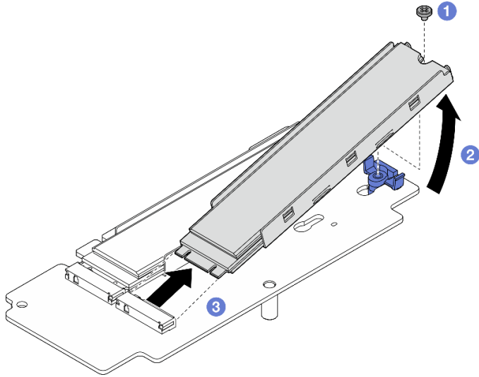
图 238. 卸下 M.2 硬盘
