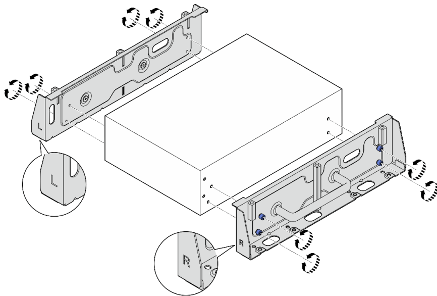
图 33. 松开指旋螺钉以卸下侧面支架
