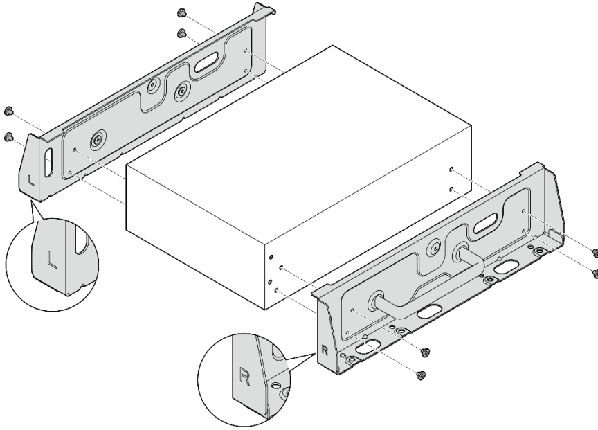
图 55. 松开螺钉以卸下侧面支架
