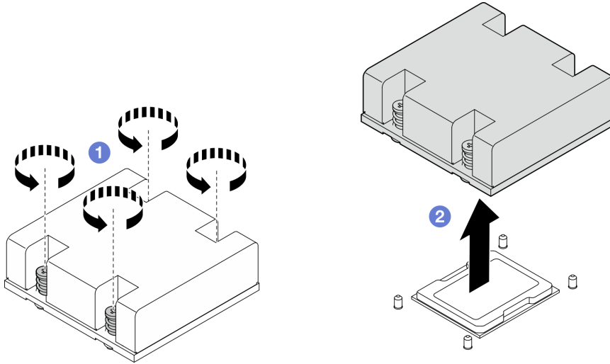
图 217. 卸下处理器散热器
