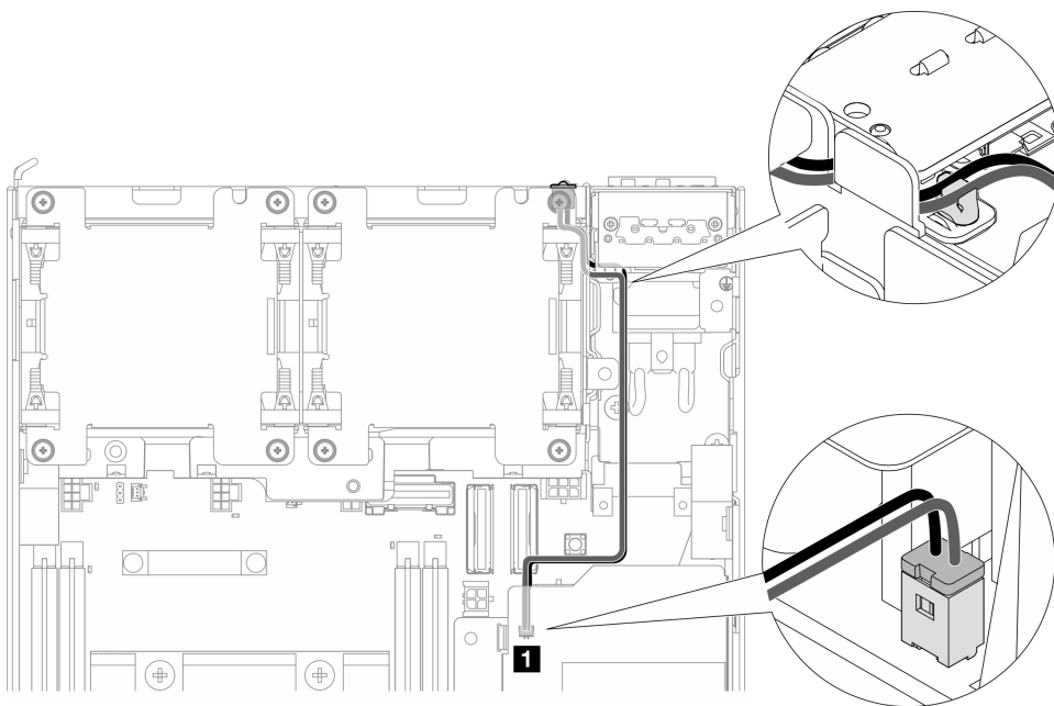
图 201. 连接到内部电源模块单元（交流 PMB）的 PMB 状态 LED 线缆
