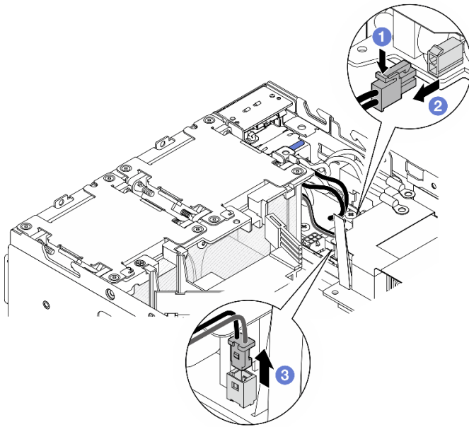
图 134. 拔下线缆
