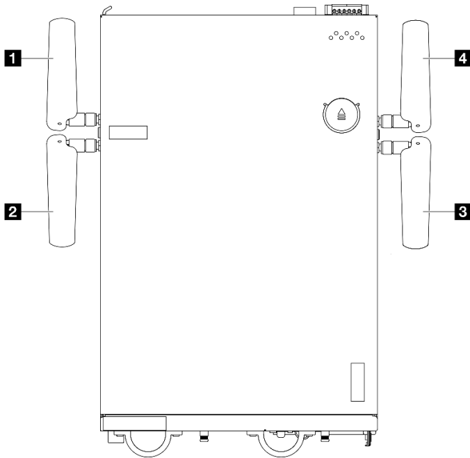
图 336. WLAN 天线的位置
