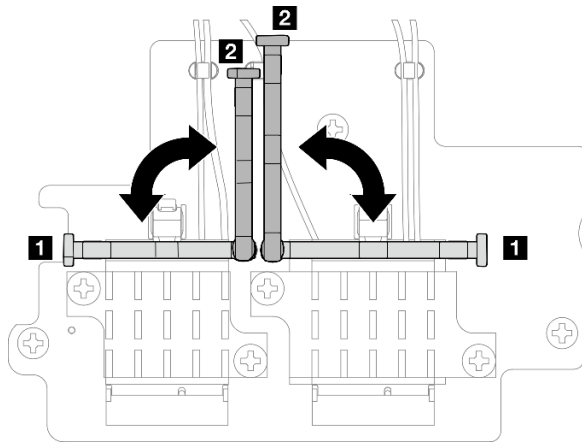
图 304. 转动线缆固定扣
