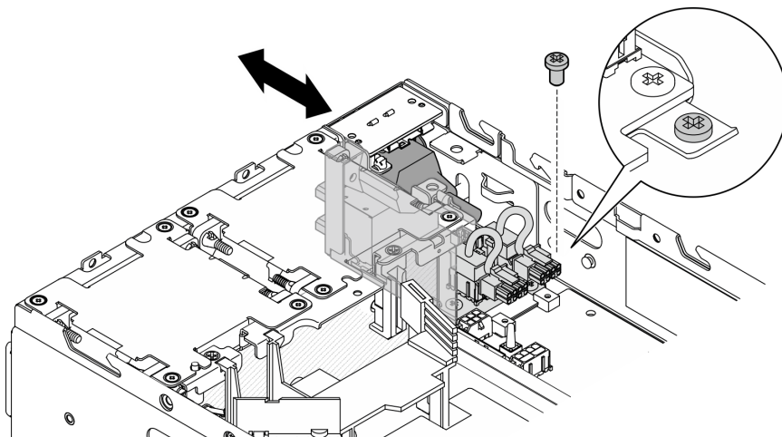
图 204. 安装 PIB 模块
