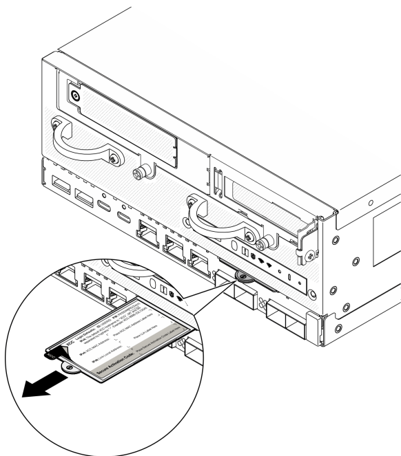
图 277. 抽取式信息卡上的 Lenovo XClarity Controller 网络访问标签
