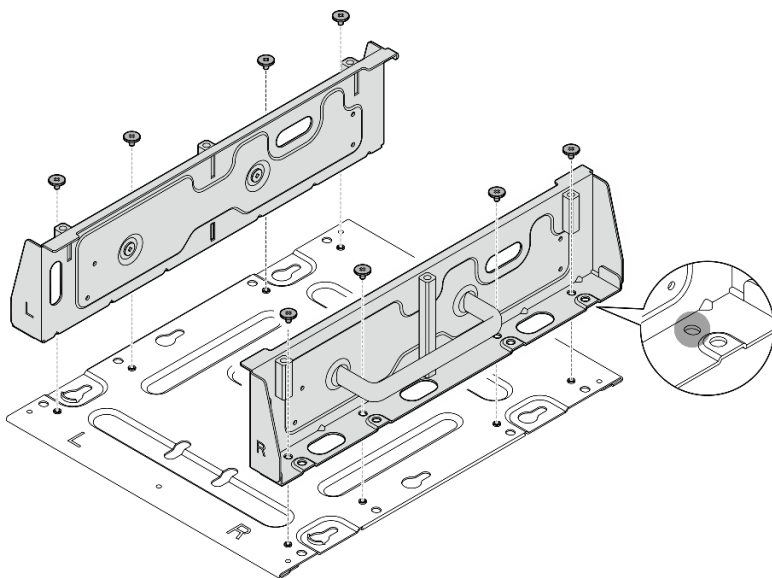
图 59. 拆卸节点支架
