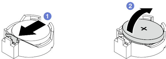
图 118. 卸下 CMOS 电池
