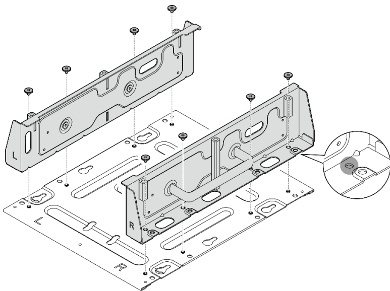
图 34. 组装节点套筒
