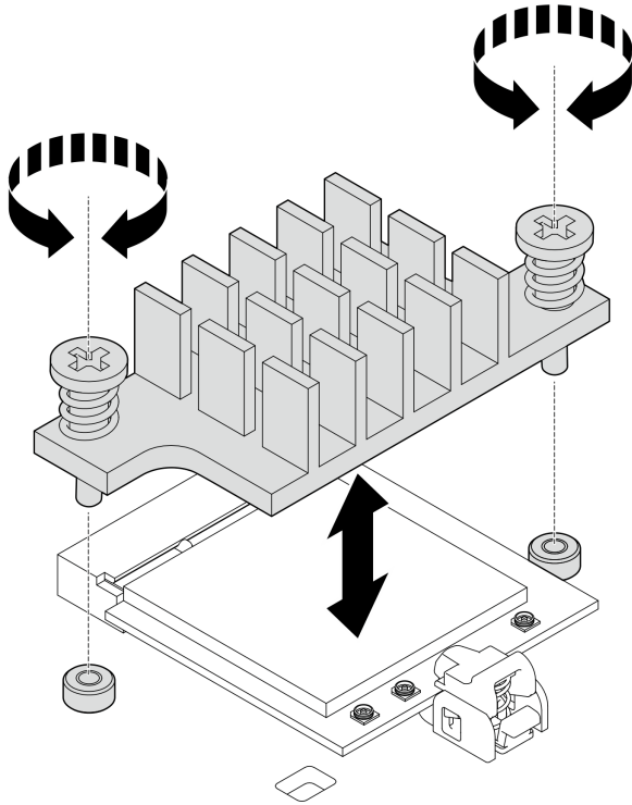
图 281. 卸下 WLAN/蓝牙模块散热器
