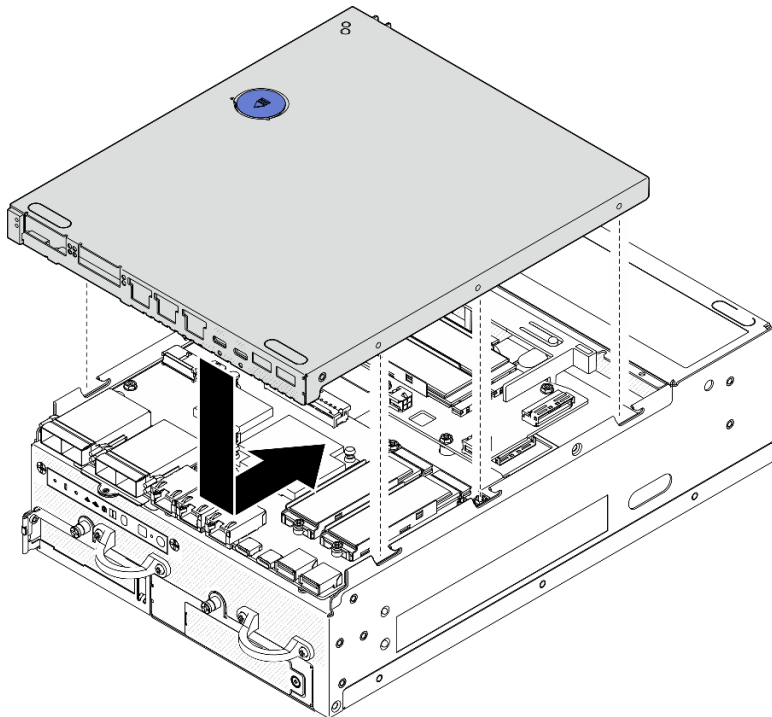
图 194. 安装底盖
