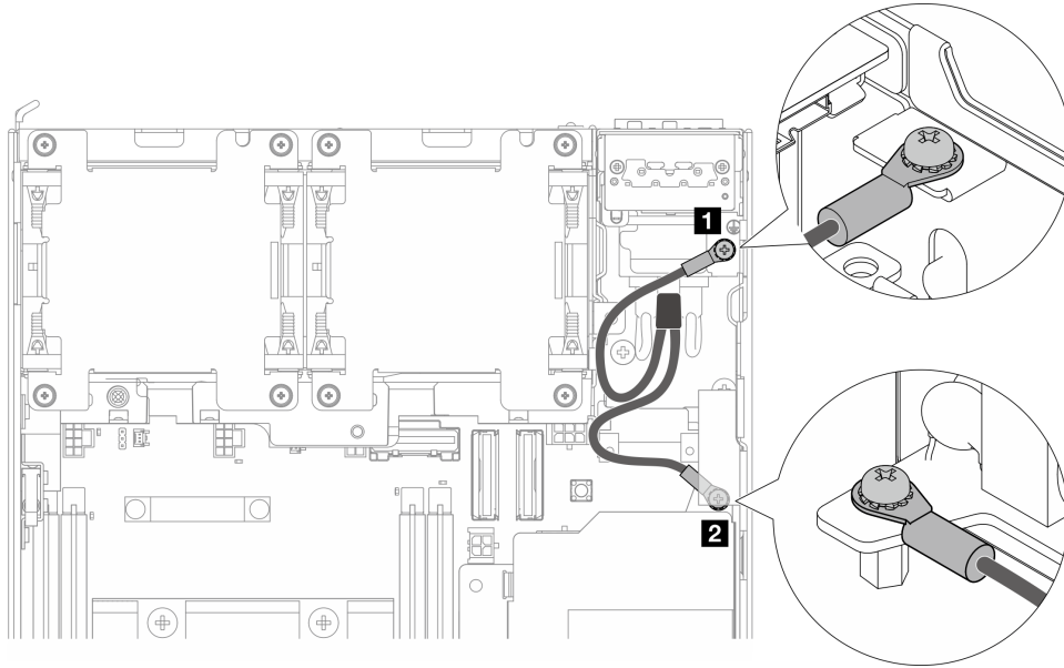
图 133. 断开接地线缆
