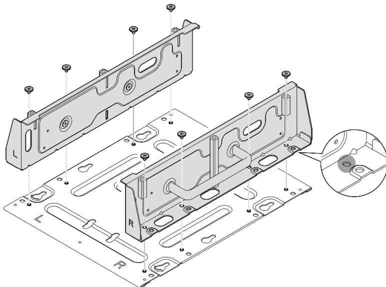
图 38. 拆卸节点支架
