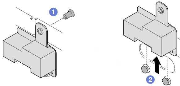
图 300. 卸下 SMA 填充件
