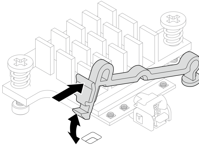
图 94. 提起线缆固定扣
