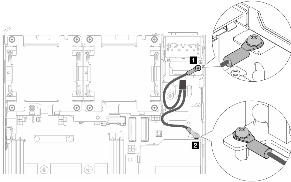
图 140. 连接接地线缆
