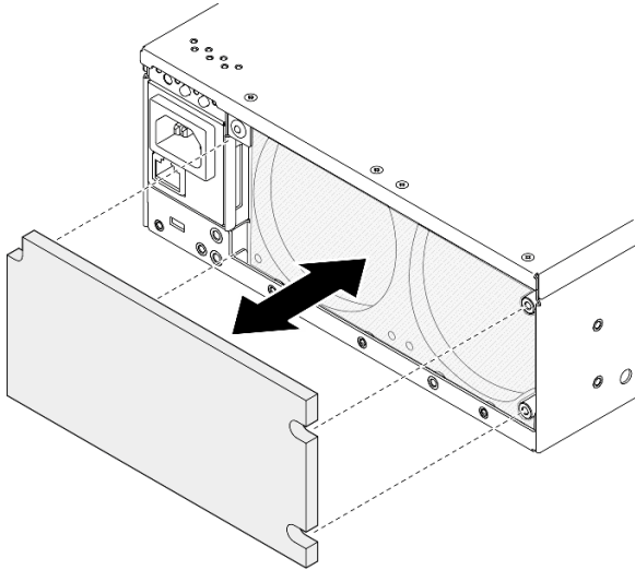
图 74. 安装灰尘过滤器
