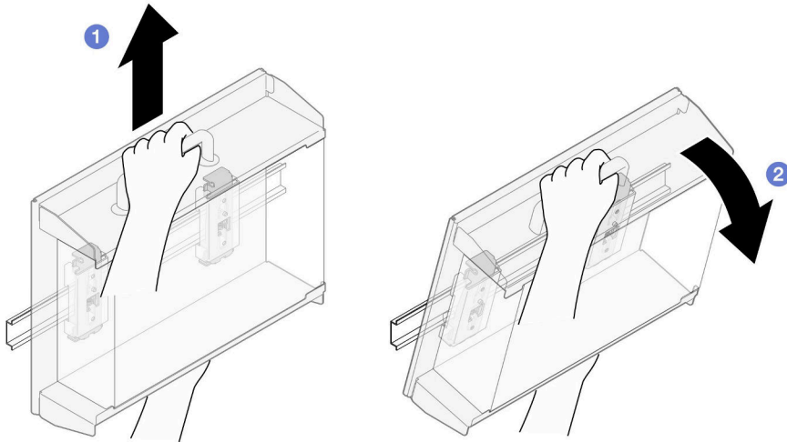
图 51. 卸下节点套筒
