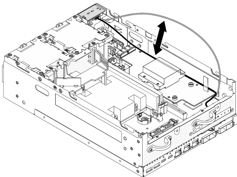
图 216. 放置信号线缆
