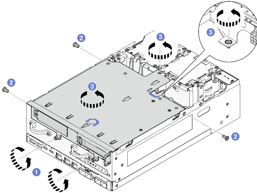
图 222. 拆卸转接卡组合件
