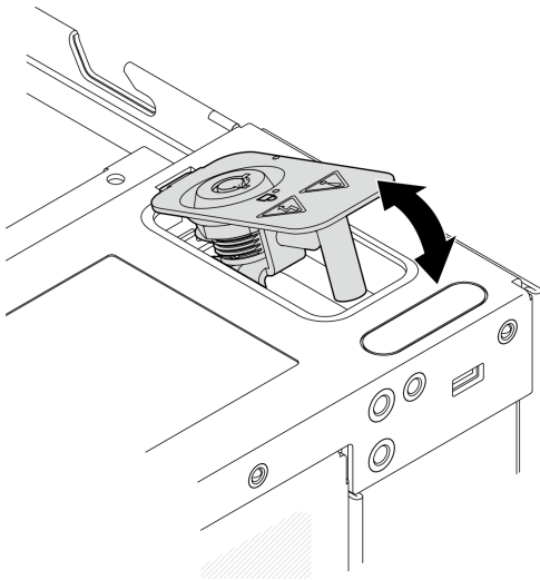
图 166. 卸下系统安全钥匙锁
