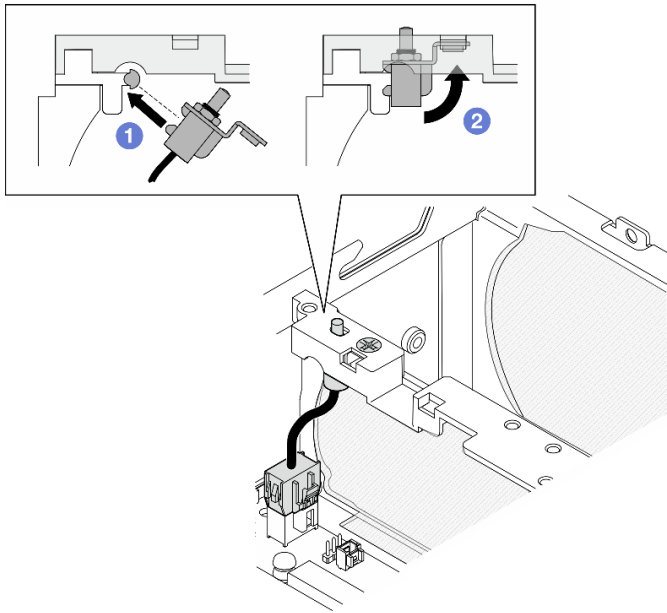
图 124. 安装带线缆的入侵感应开关
