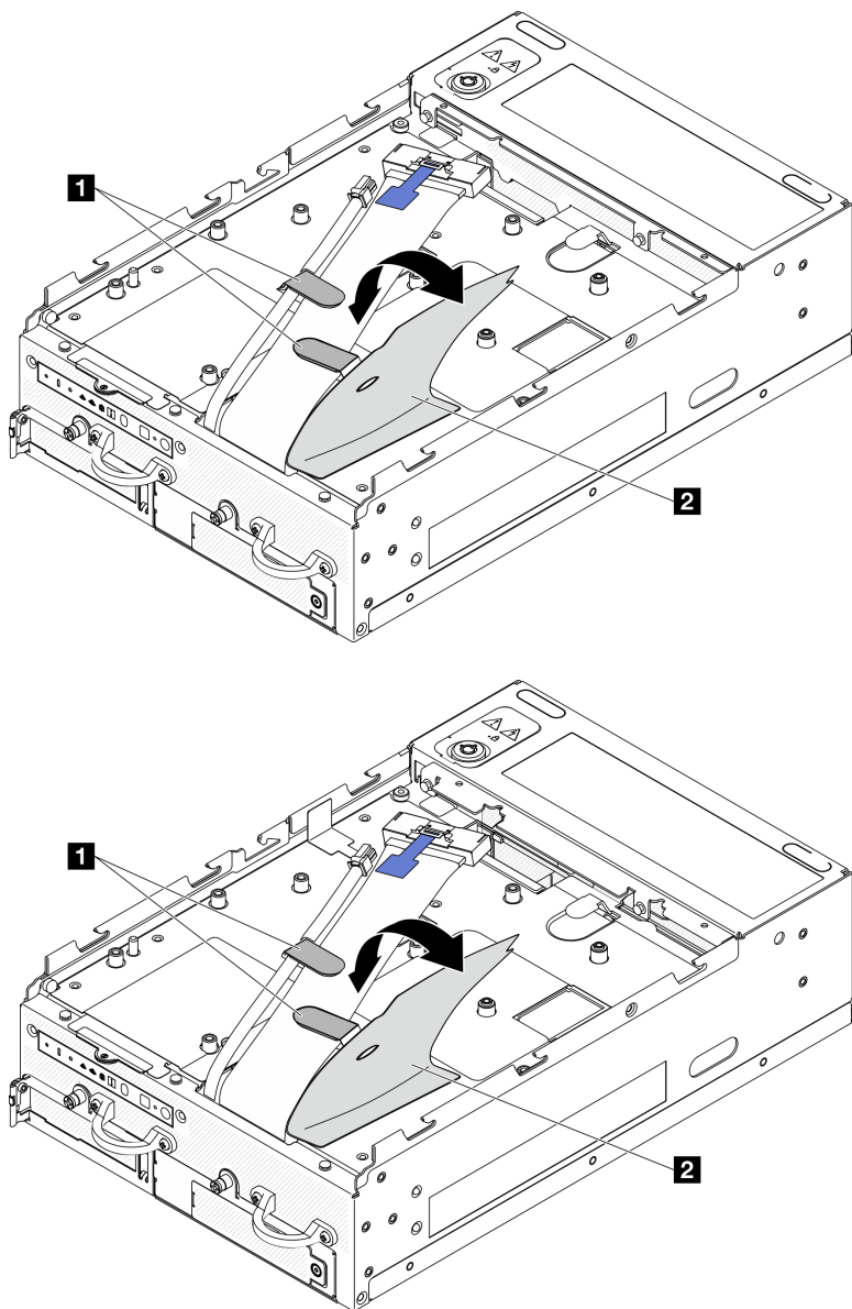
图 156. I/O 板线缆布放
