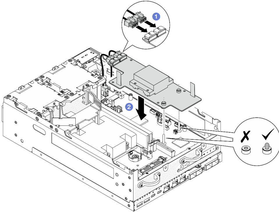
图 212. 安装电源模块板
