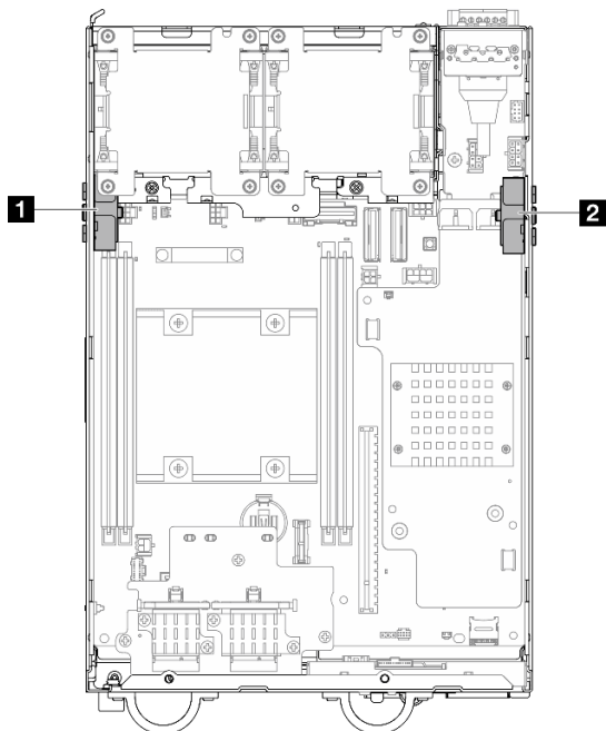
图 323. SMA 组合件位置
