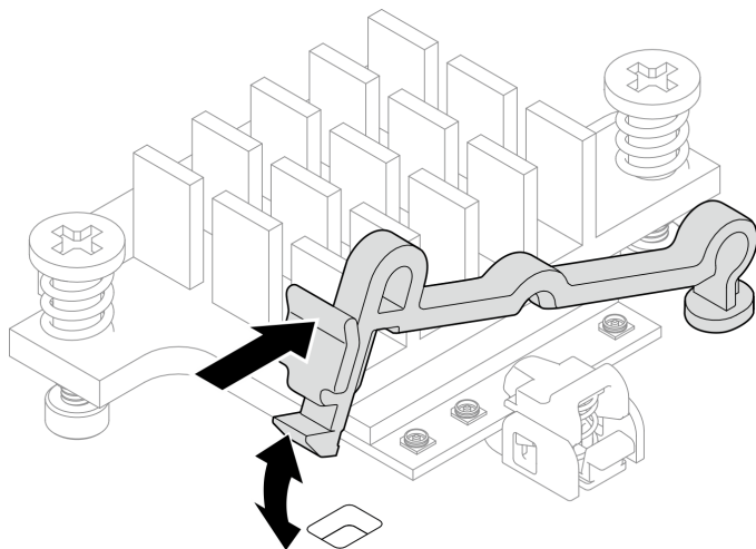
图 293. 插入线缆固定扣
