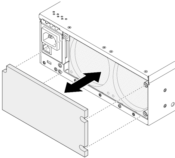
图 73. 卸下灰尘过滤器
