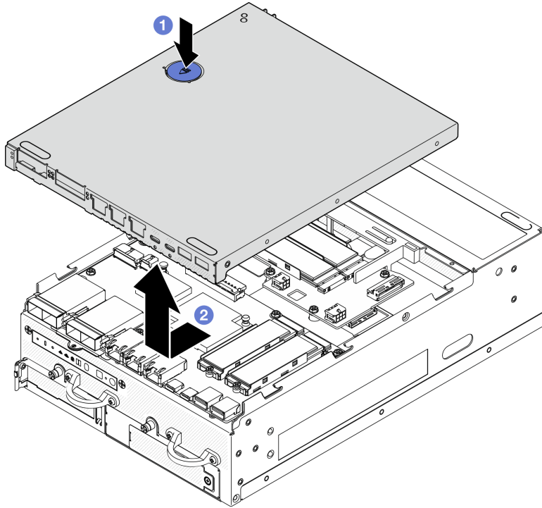
图 191. 卸下底盖
