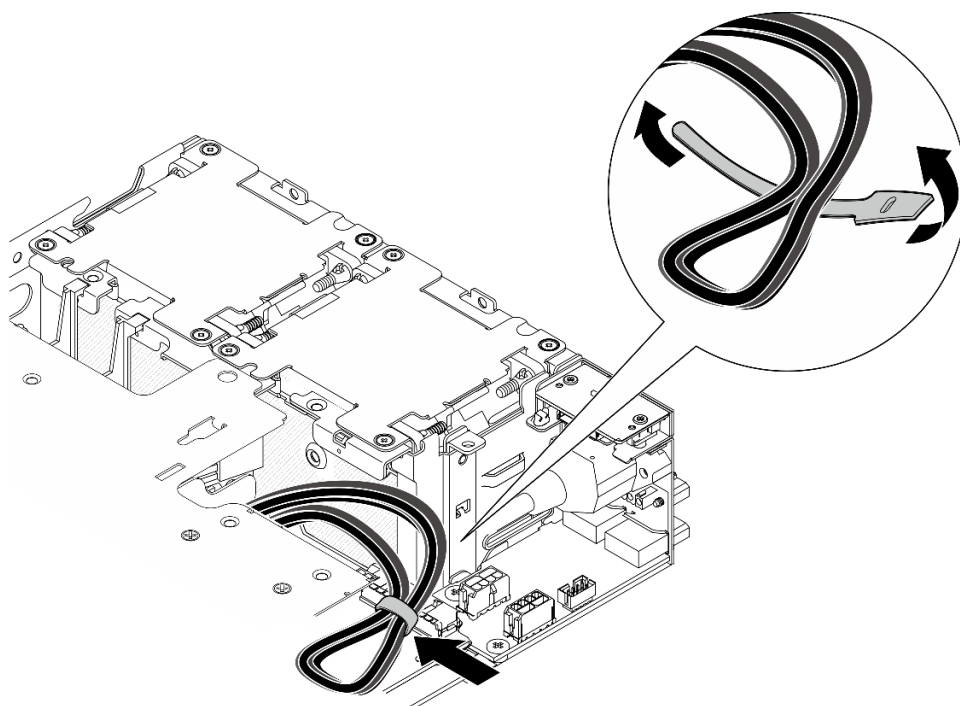
图 269. 转接卡组合件的线缆布放
