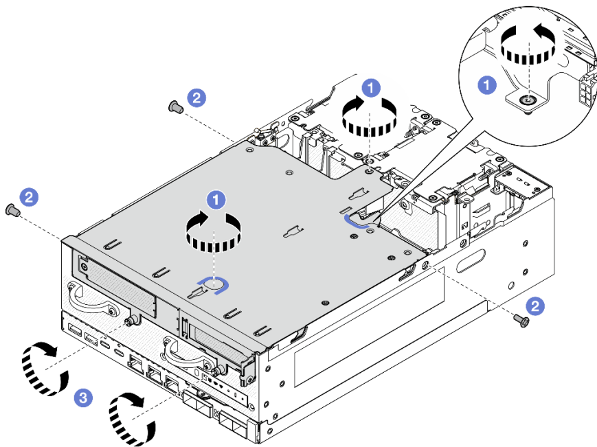
图 268. 固定转接卡组合件
