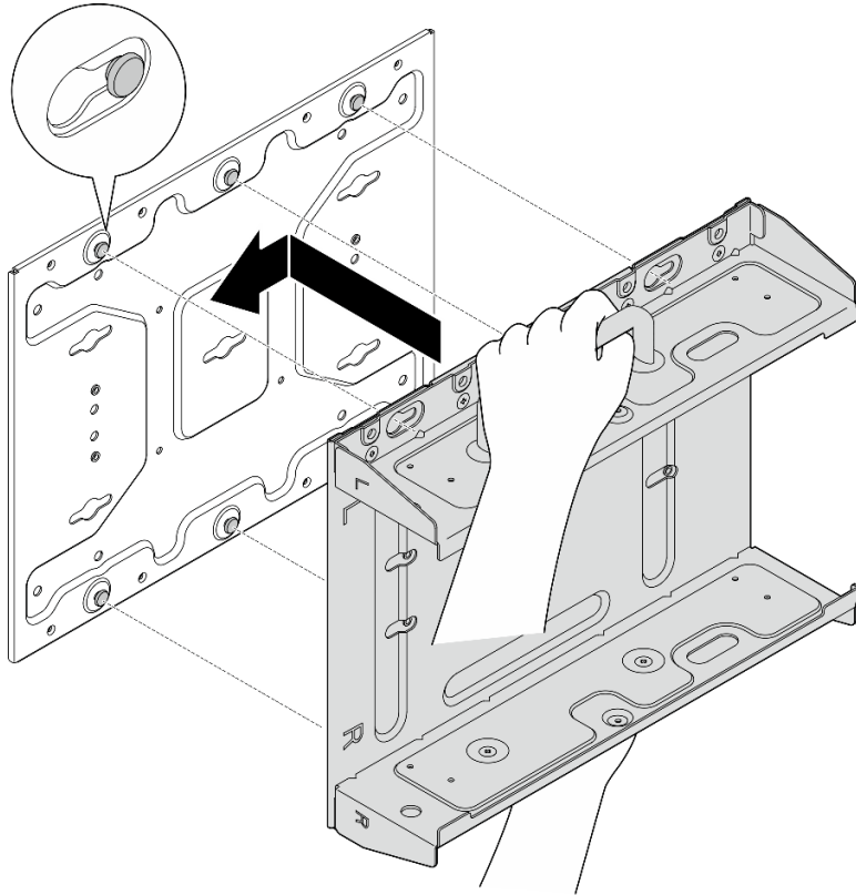
图 35. 组装节点套筒
