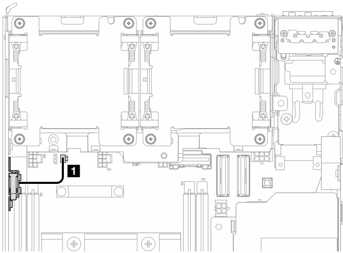
图 142. 顶部入侵感应开关线缆布放
