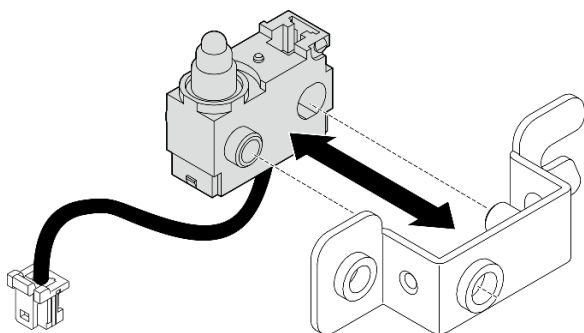
图 145. 将入侵感应开关插入支架
