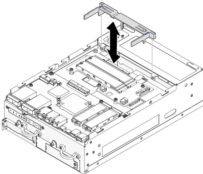
图 82. 卸下导风罩
