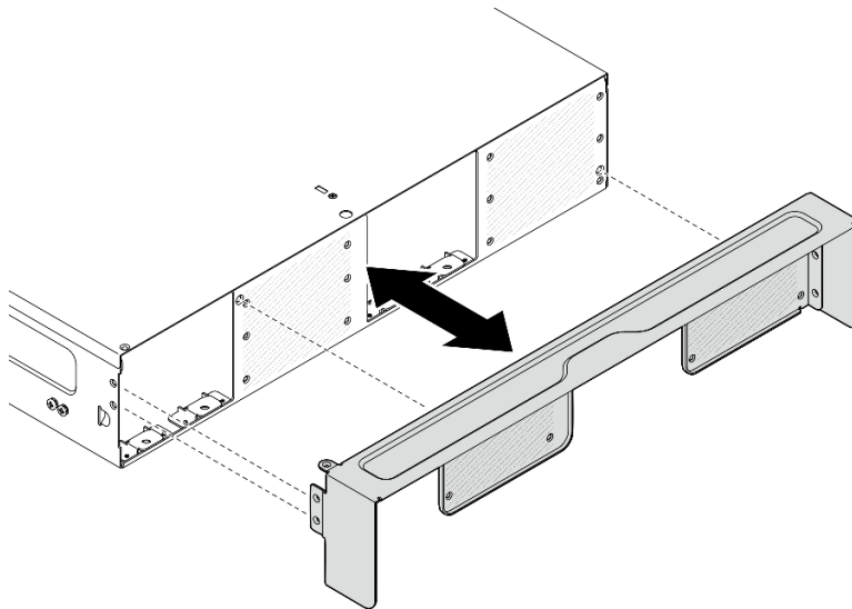
图 11. 卸下装运支架
