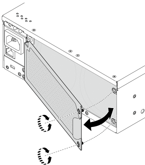
图 72. 卸下挡板
