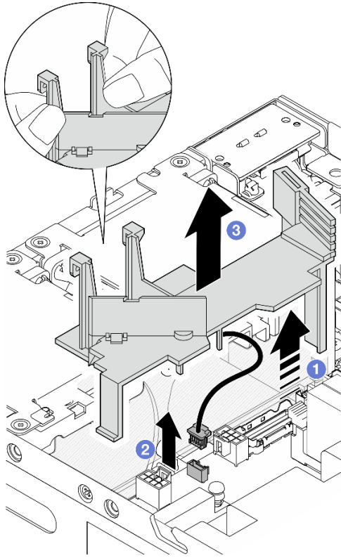
图 87. 卸下导风罩
