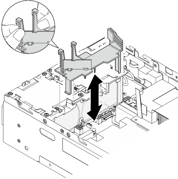
图 86. 卸下导风罩
