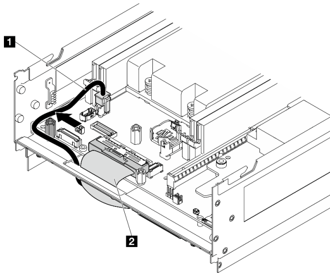
图 158. I/O 板线缆布放
