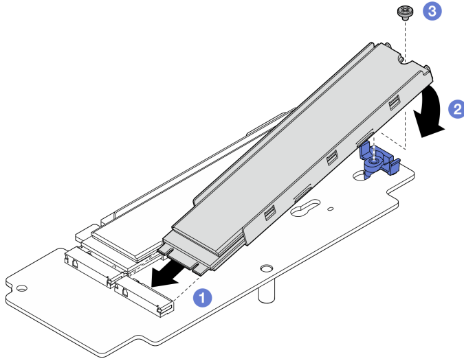
图 241. 安装 M.2 硬盘
