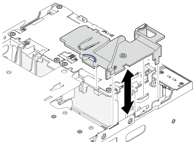
图 84. 卸下导风罩
