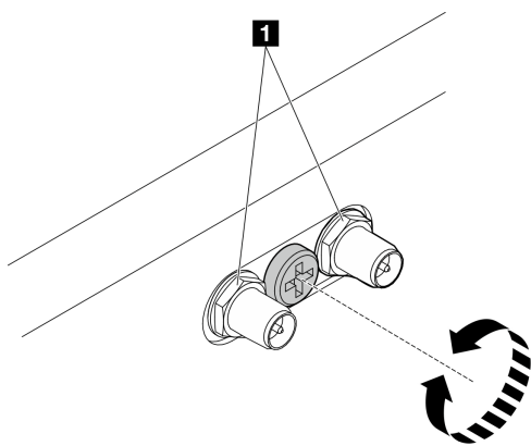
图 299. 缩短 SMA 接口
