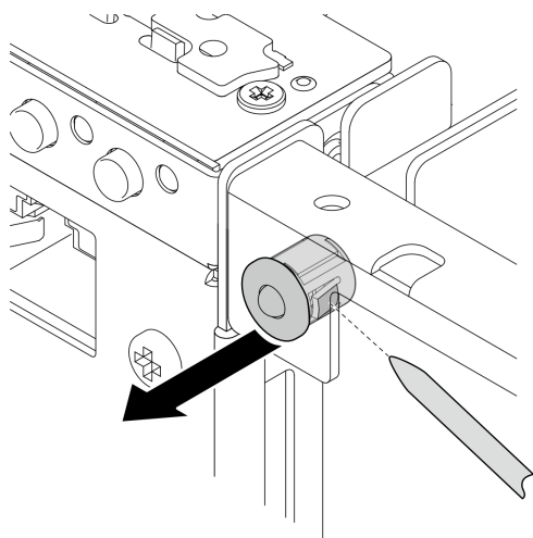
图 198. 拔下 PMB 状态 LED 线缆
