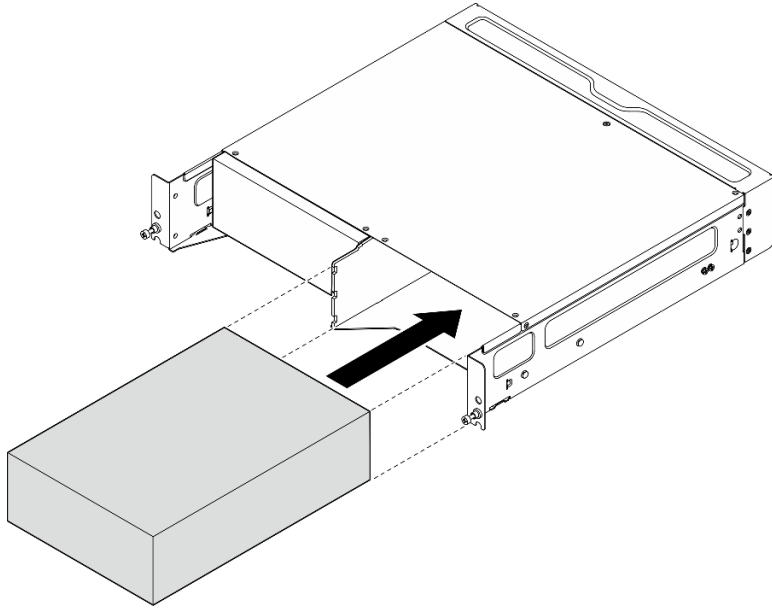
图 22. 安装节点
