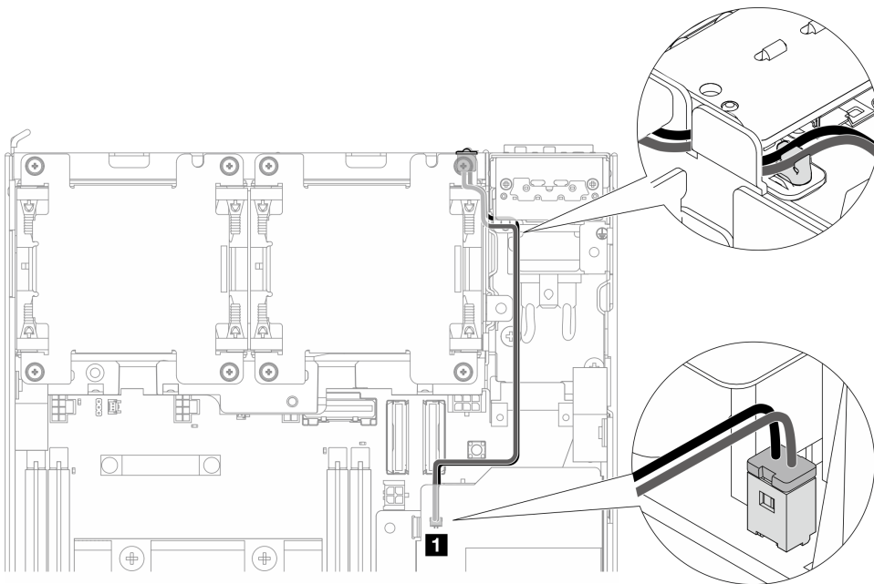
图 197. 连接到内部电源模块单元（交流 PMB）的 PMB 状态 LED 线缆
