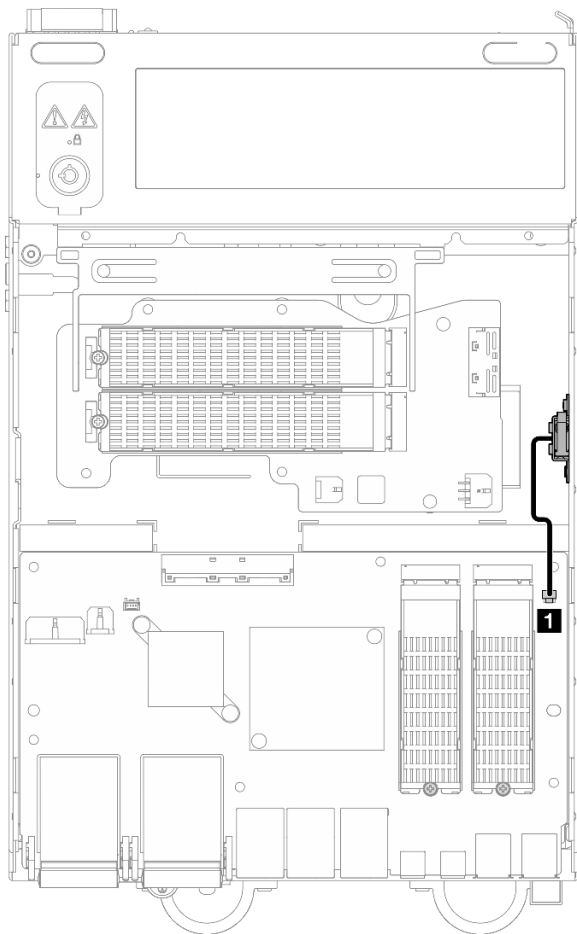
图 148. 底部入侵感应开关线缆布放
