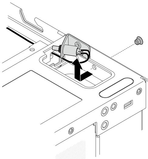
图 168. 卸下带线缆的锁定位置开关
