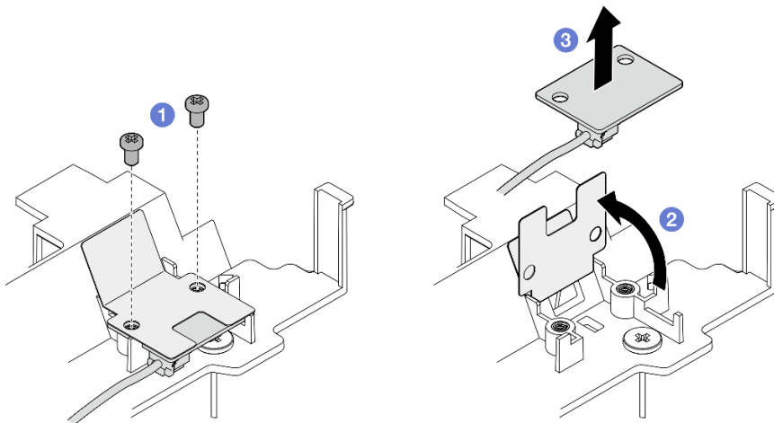
图 88. 卸下气流传感器板
