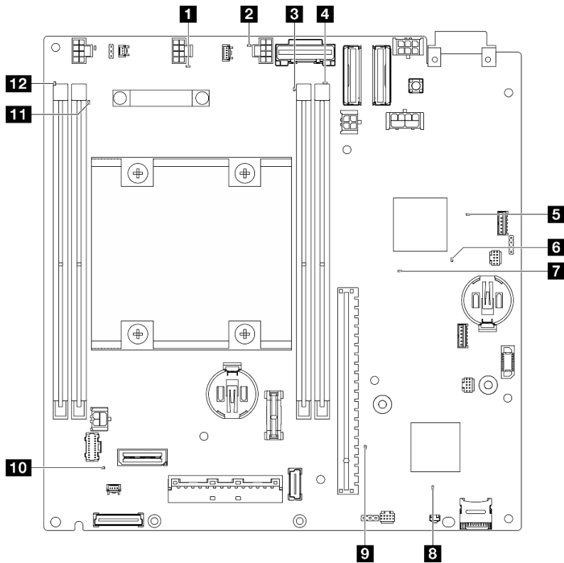
图 351. 主板 LED
