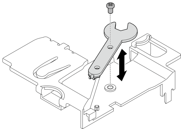
图 298. 取下扳手
