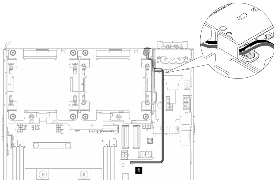
图 215. PMB LED 线缆
