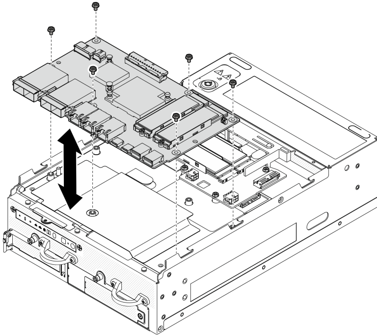
图 160. 安装 I/O 模块板
