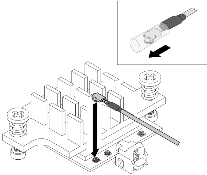
图 331. 连接线缆
