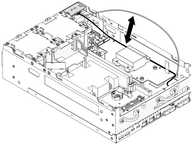
图 207. 放置信号线缆
