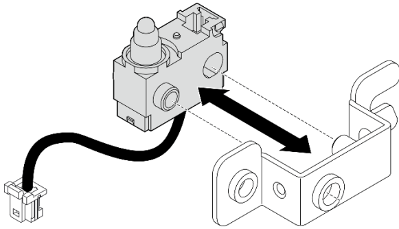
图 144. 从支架上拆下入侵感应开关
