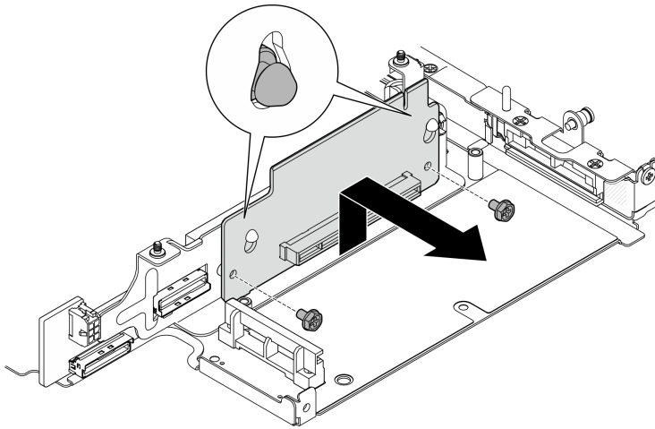
图 237. 卸下转接卡
