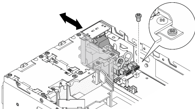
图 202. 卸下直流 PIB 模块
