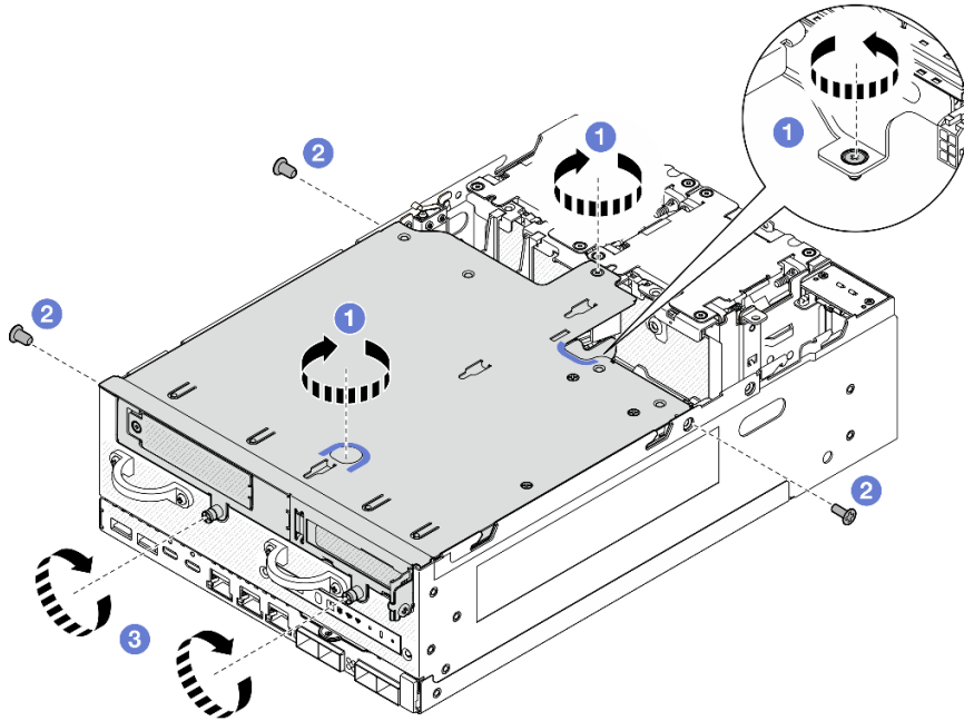
图 261. 固定转接卡组合件
