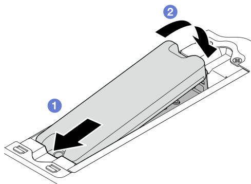
图 259. 安装 位置跟踪模块
