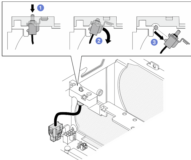
图 123. 卸下风扇方向开关
