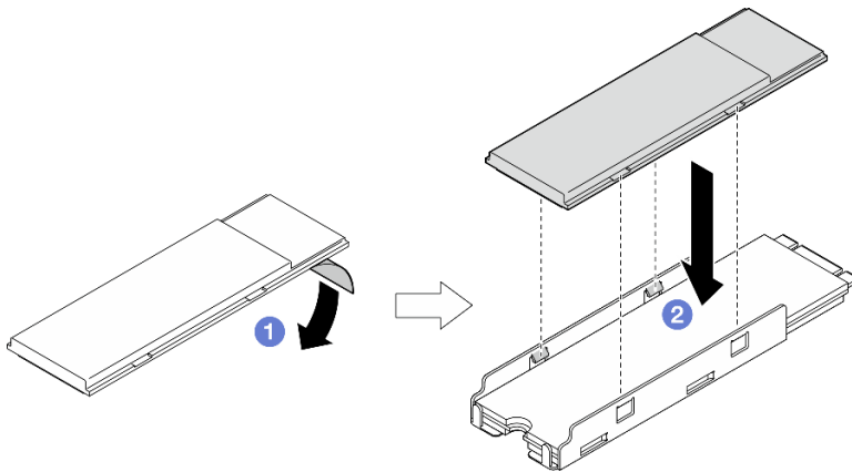
图 175. 安装 M.2 散热器
