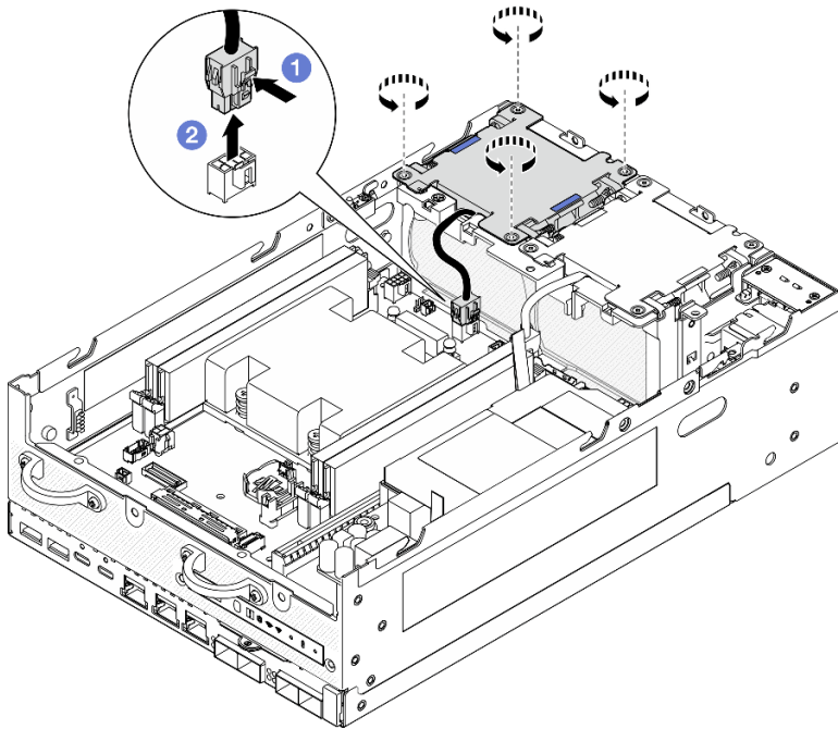
图 126. 卸下风扇模块
