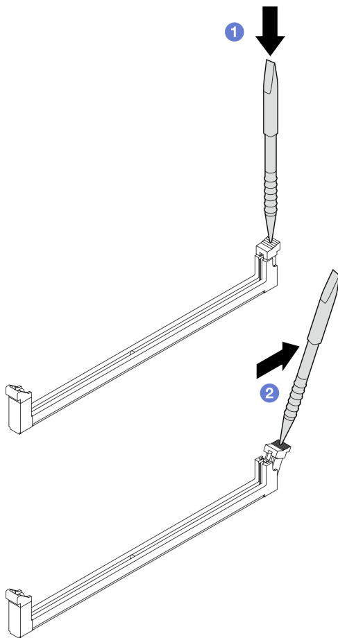
图 180. 打开固定夹
