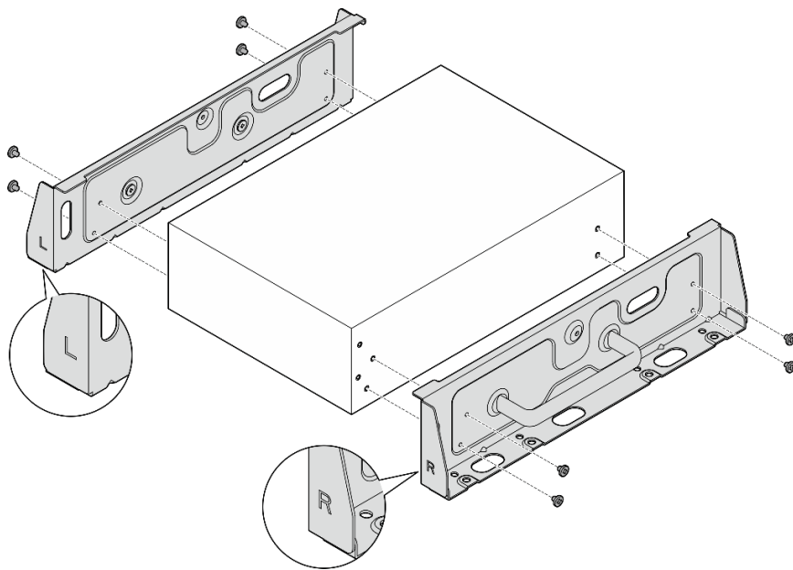
图 40. 用螺钉安装侧面支架
