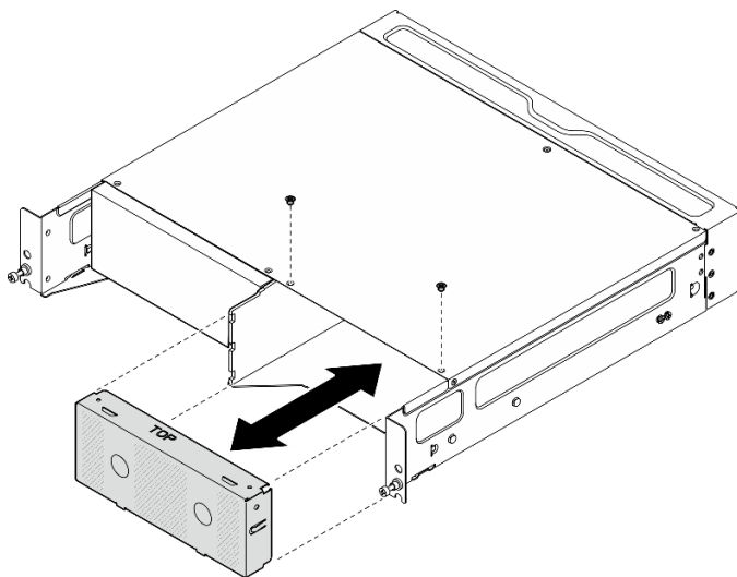
图 23. 安装节点填充件
