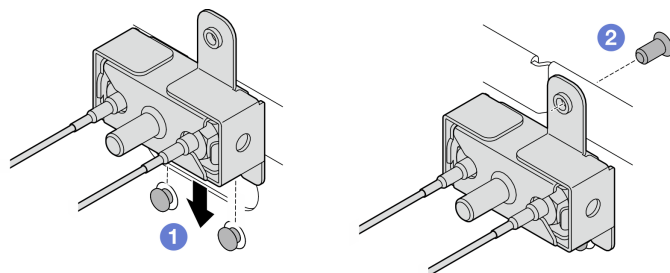
图 326. 安装 SMA 组合件
