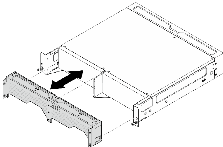
图 24. 安装装运支架
