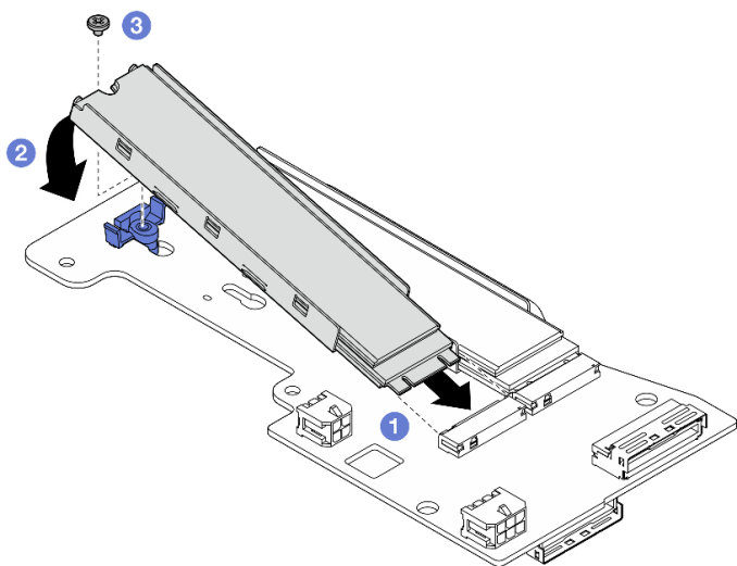
图 246. 安装 M.2 硬盘
