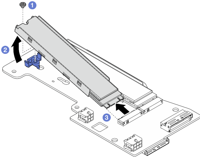
图 112. 卸下 M.2 硬盘
