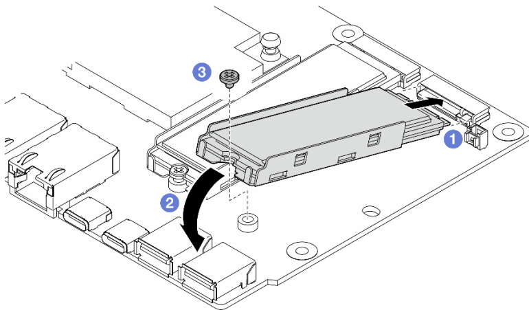
图 162. 安装 M.2 硬盘
