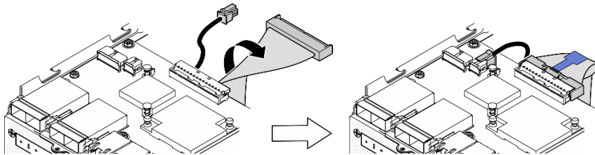
图 161. 连接 I/O 板线缆
