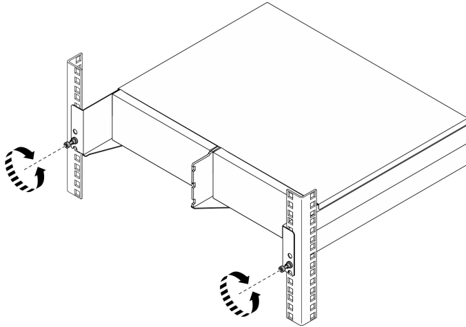
图 7. 使机柜与机架脱离
