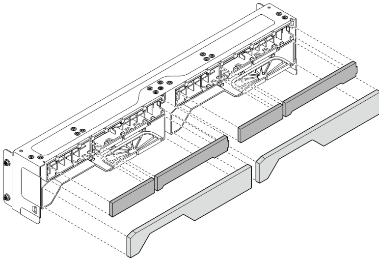
图 69. 安装灰尘过滤器
