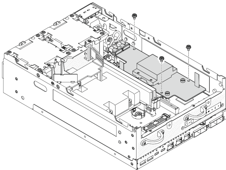
图 214. 固定电源模块板
