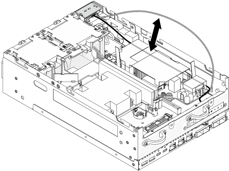
图 137. 放置信号线缆
