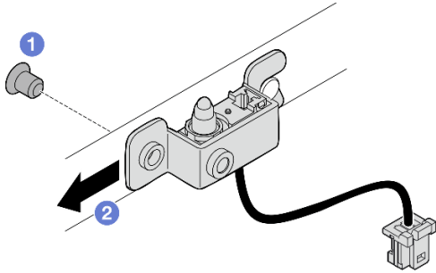
图 149. 卸下带线缆的入侵感应开关
