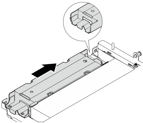
图 257. 安装 位置跟踪模块仓
