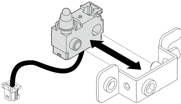
图 150. 从支架上拆下入侵感应开关
