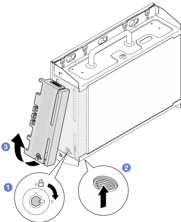
图 26. 卸下安全挡板
