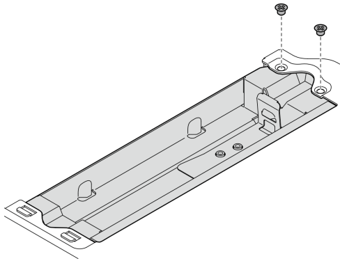
圖例 258. 安裝地理位置追蹤模組盒
