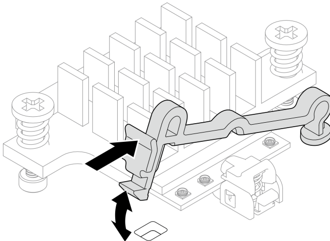
圖例 94. 提起纜線固定器
