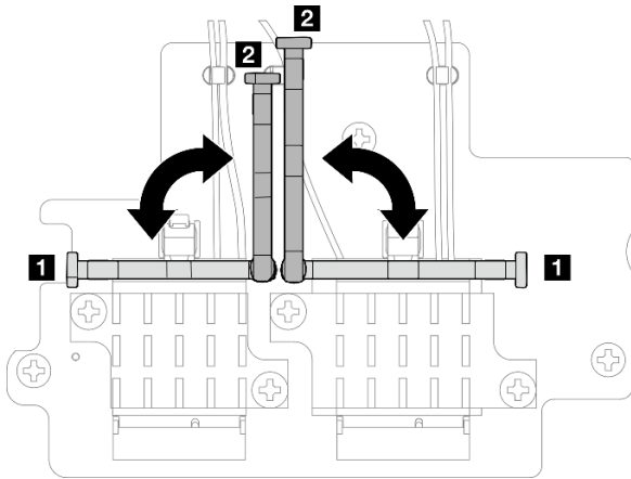
圖例 108. 轉動纜線固定器
