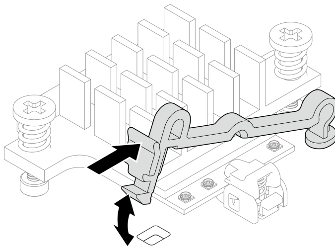
圖例 293. 插入纜線固定器
