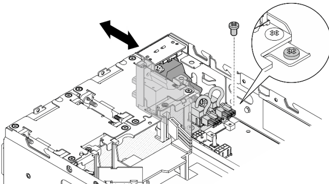
圖例 202. 卸下 DC PIB 模組
