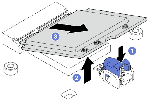
圖例 282. 卸下 WLAN/藍牙模組
