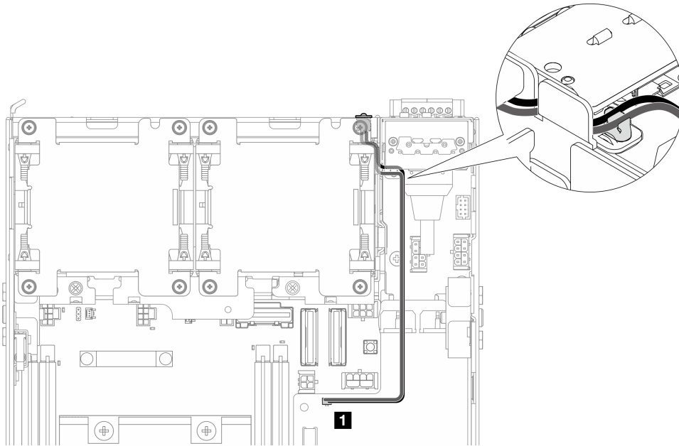
圖例 196. 連接到 DC 電源模組板 (DC PMB) 的 PMB 狀態 LED 纜線
