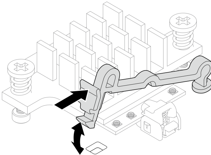
圖例 312. 提起纜線固定器
