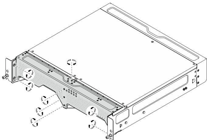
圖例 66. 鬆開螺絲
