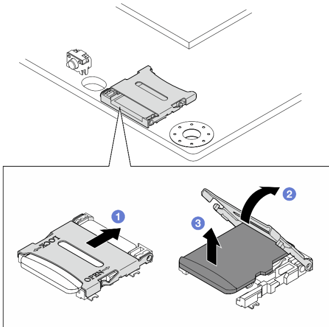
圖例 182. 卸下 MicroSD 卡
