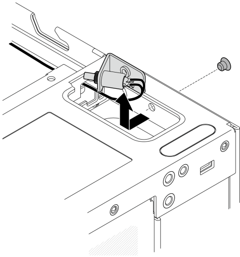
圖例 168. 卸下鎖定位置開關及纜線
