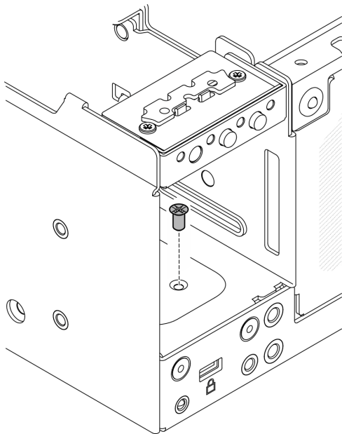
圖例 172. 鎖緊螺絲
