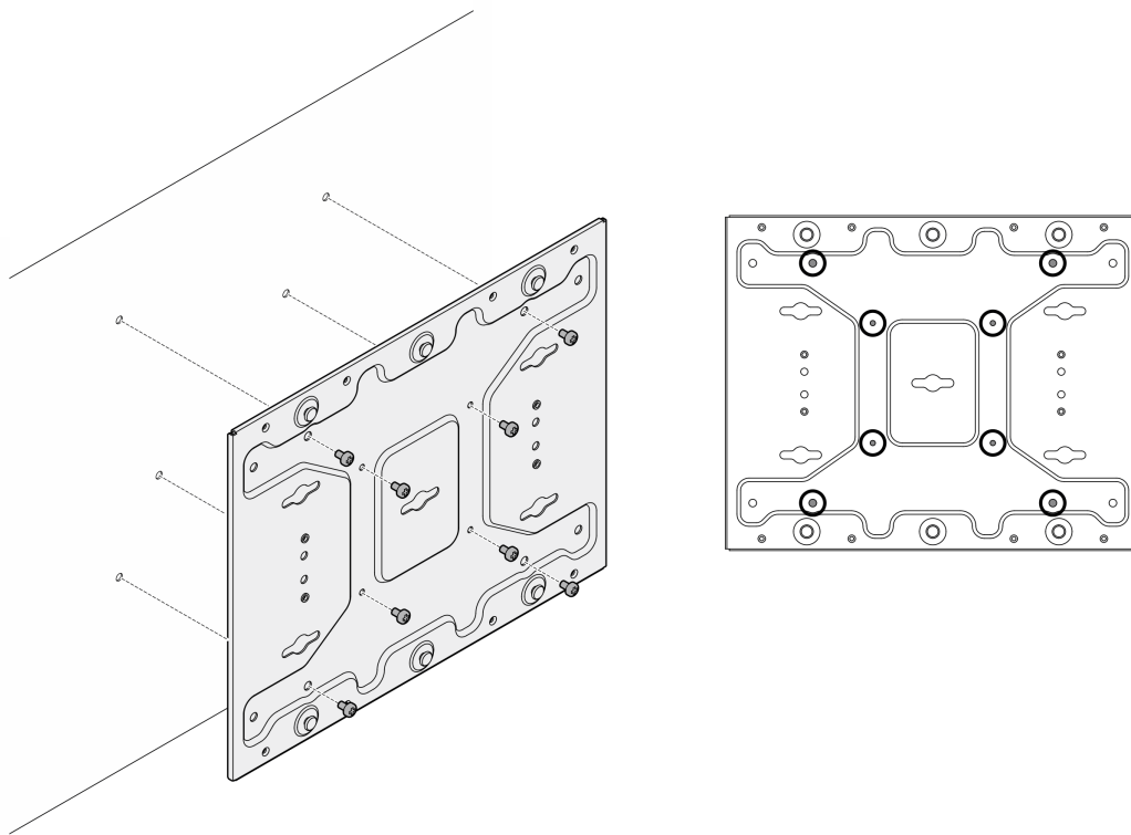
圖例 29. 卸下壁掛板
