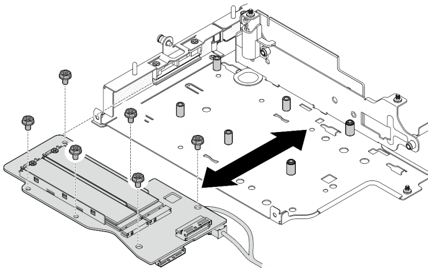
圖例 225. 卸下 M.2 含纜線配接卡
