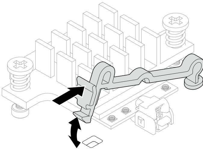
圖例 316. 插入纜線固定器
