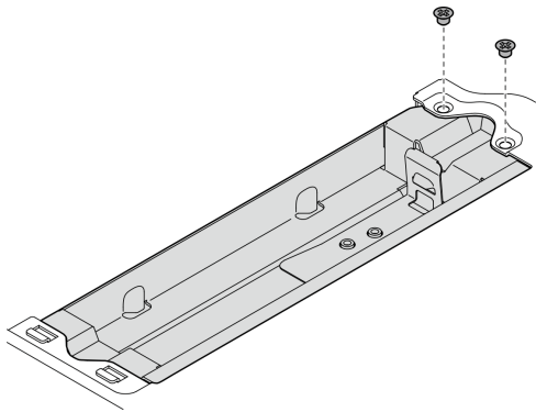
圖例 232. 卸下地理位置追蹤模組盒
