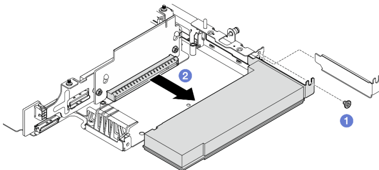
圖例 239. 卸下 PCIe 配接卡
