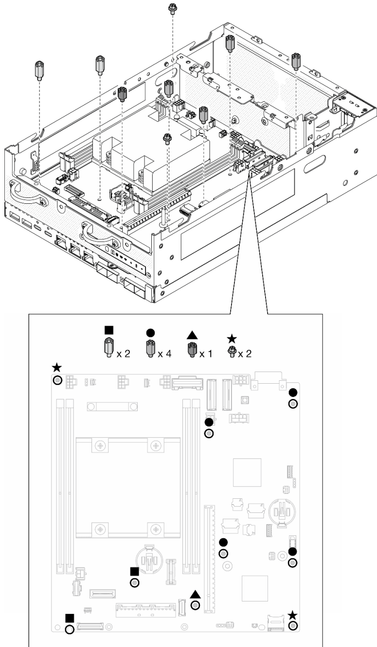
圖例 275. 主機板上的螺絲和支座
