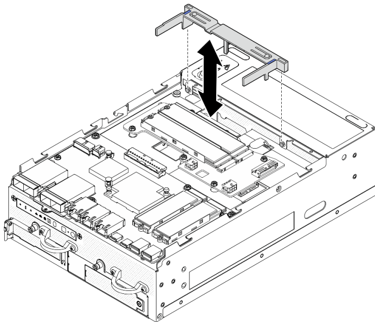
圖例 82. 卸下空氣擋板
