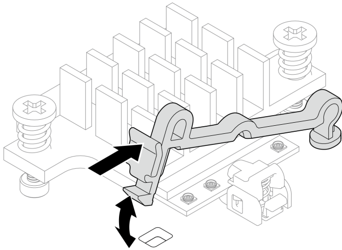
圖例 328. 提起纜線固定器
