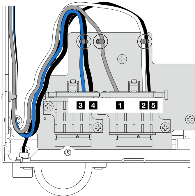
圖例 334. 無線配接卡的纜線佈線
