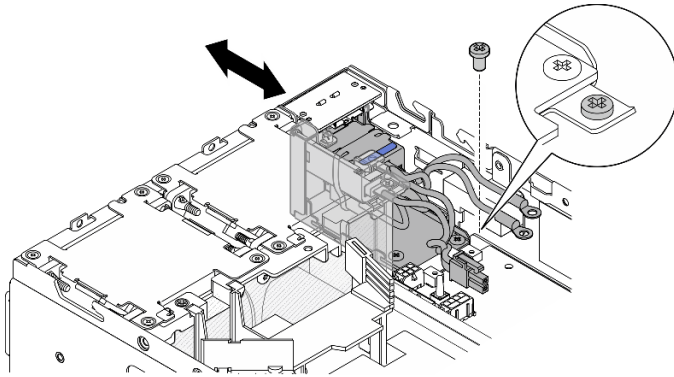
圖例 206. 安裝 PIB 模組
