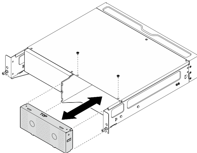
圖例 5. 安裝節點填充板
