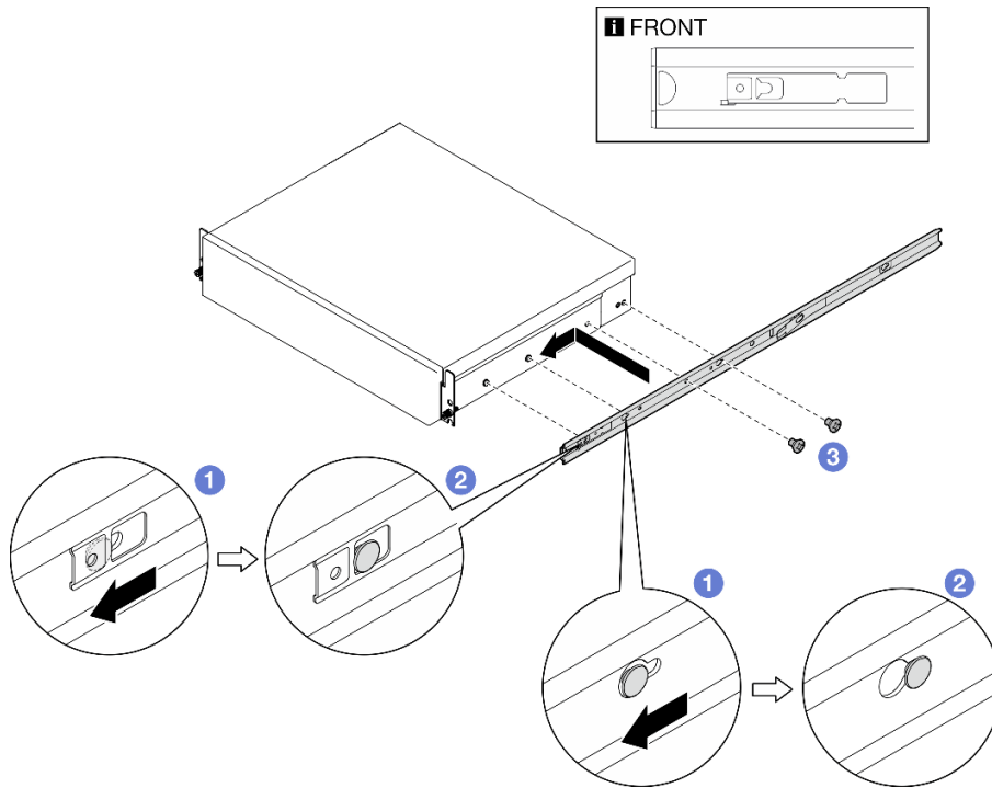
圖例 16. 安裝內滑軌
