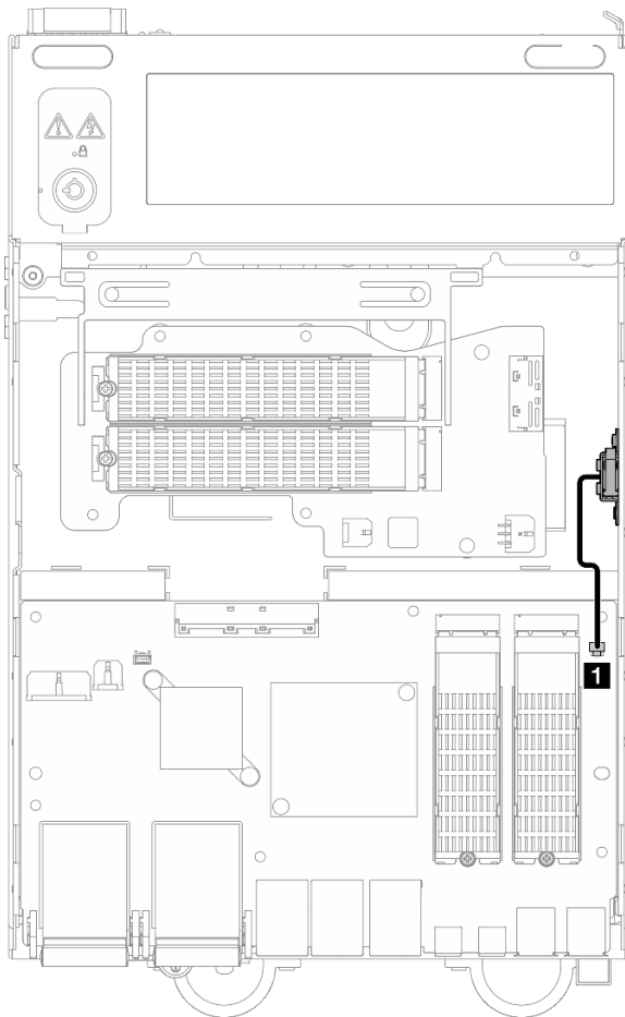
圖例 148. 底部入侵開關纜線佈線
