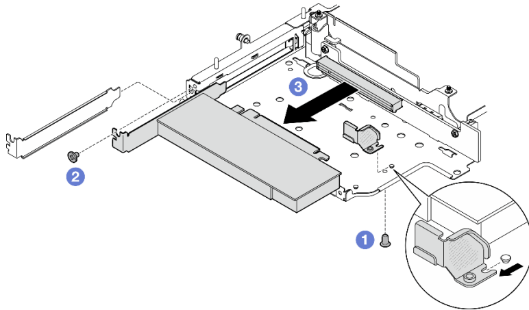
圖例 227. 卸下 PCIe 配接卡
