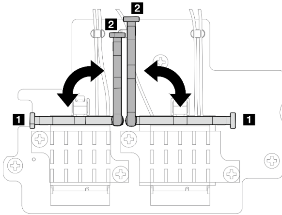
圖例 315. 轉動纜線固定器
