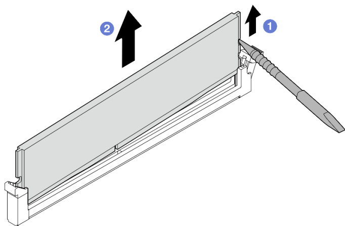
圖例 178. 卸下記憶體模組
