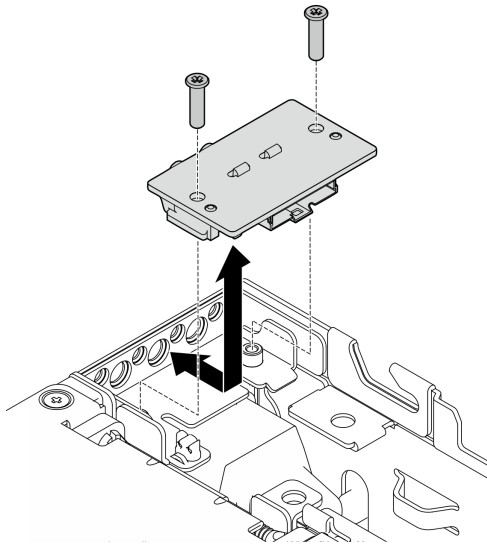
圖例 221. 安裝後方操作面板
