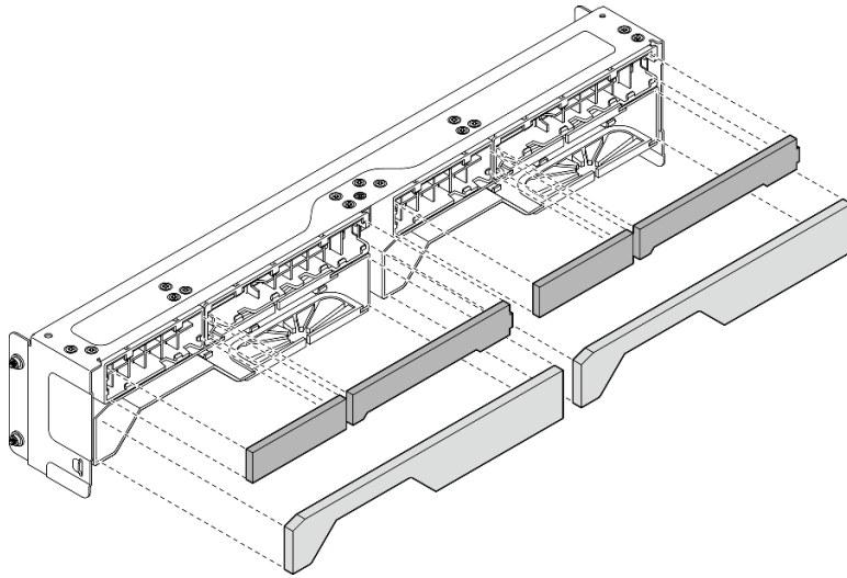
圖例 68. 卸下灰塵過濾器
