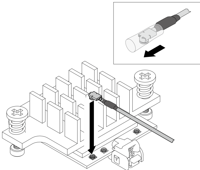
圖例 291. 連接纜線
