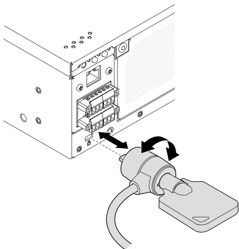
圖例 163. 卸下 Kensington 安全鎖
