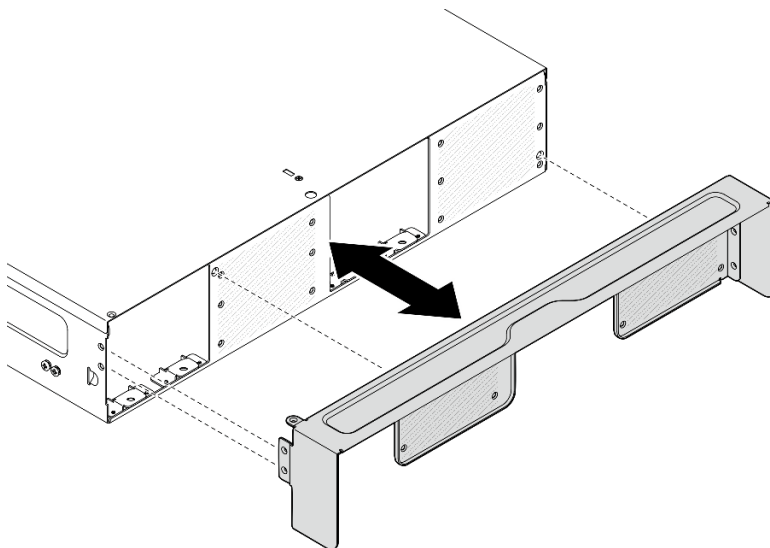
圖例 11. 卸下出貨托架
