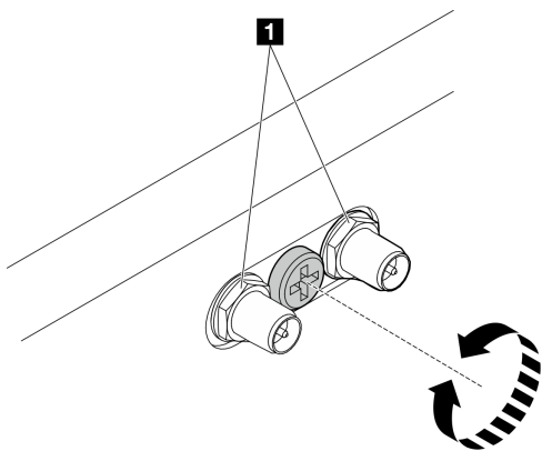
圖例 310. 縮短 SMA 接頭
