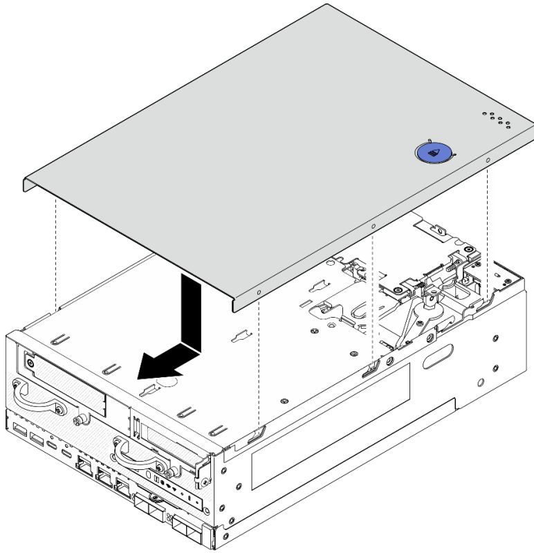
圖例 188. 安裝上蓋
