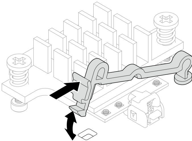
圖例 98. 插入纜線固定器
