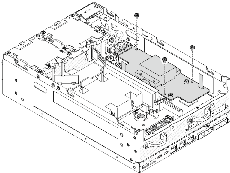
圖例 209. 鬆開螺絲
