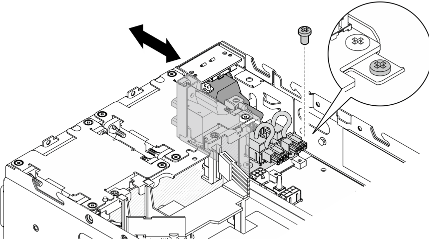
圖例 204. 安裝 PIB 模組
