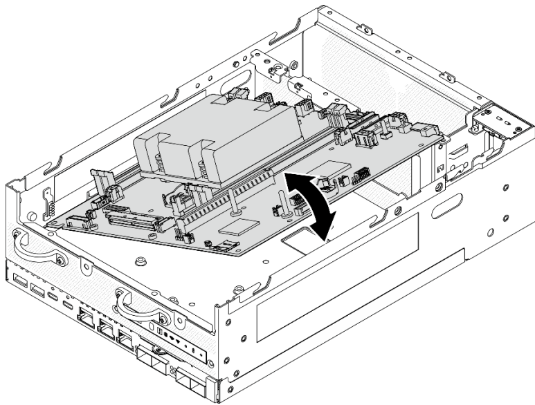
圖例 274. 安裝主機板
