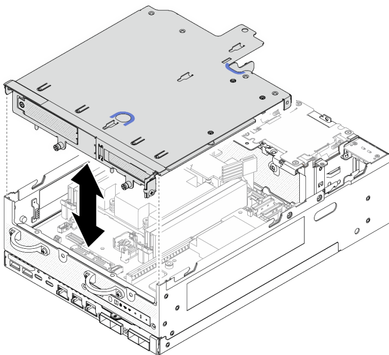
圖例 266. 放下擴充卡組件
