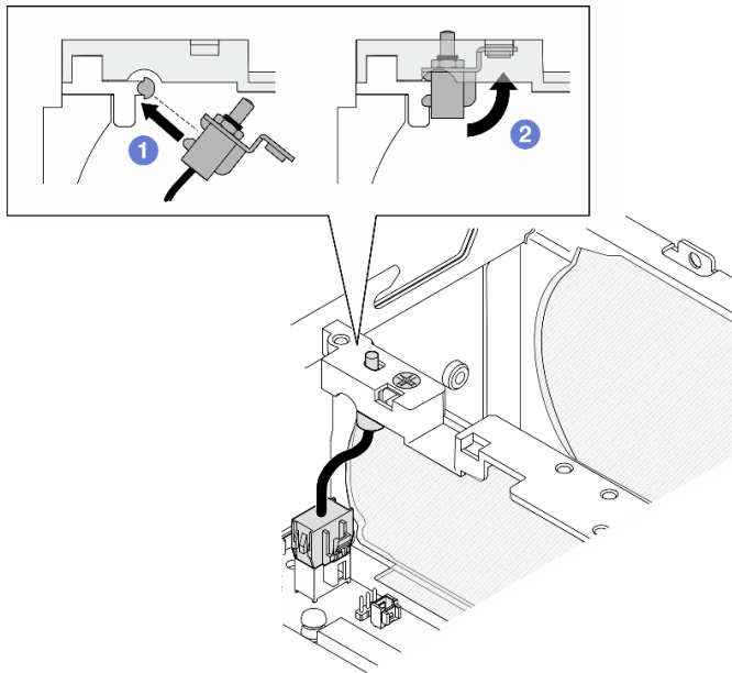
圖例 124. 安裝入侵開關及纜線
