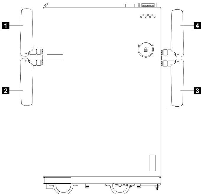
圖例 295. WLAN 天線的位置
