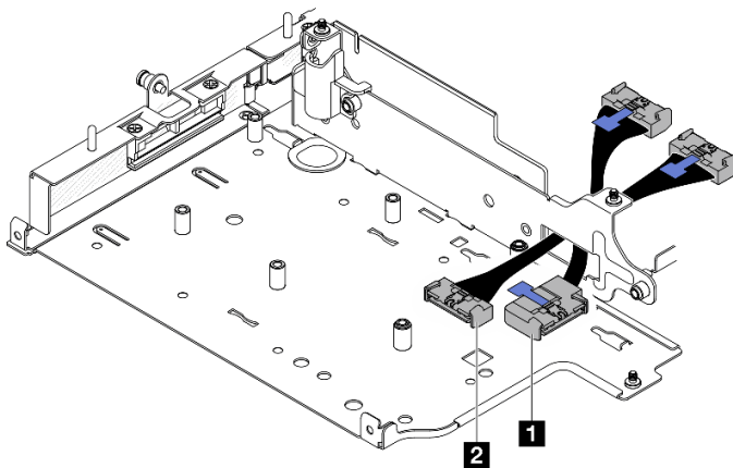
圖例 247. M.2 含纜線配接卡信號線
