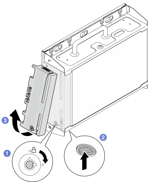
圖例 26. 卸下安全擋板
