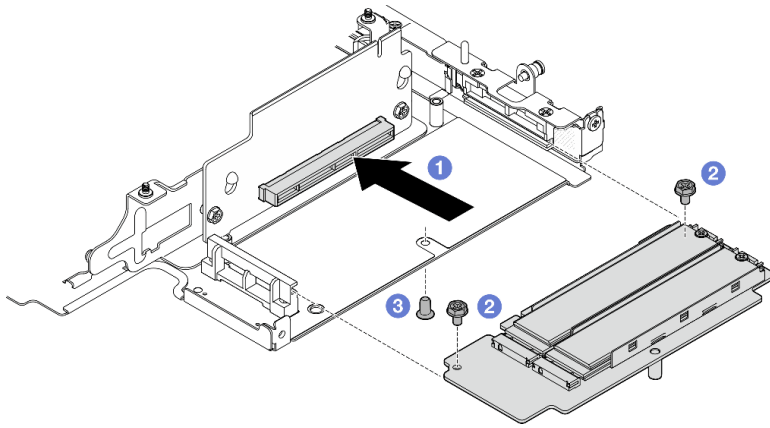
圖例 243. 安裝 M.2 配接卡
