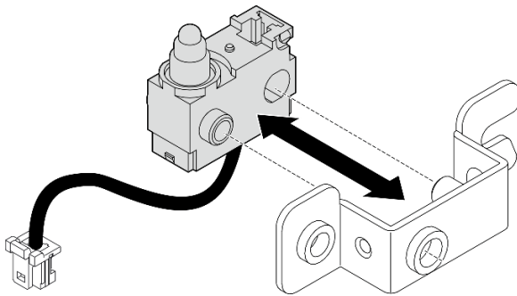
圖例 150. 將入侵開關與托架分開
