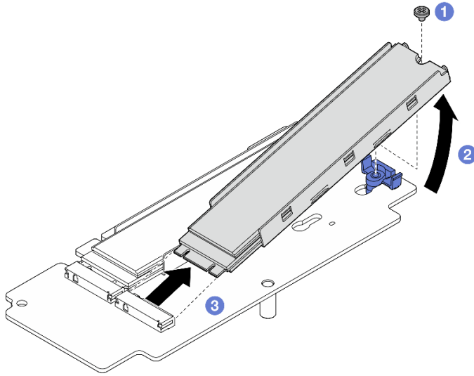
圖例 238. 卸下 M.2 硬碟
