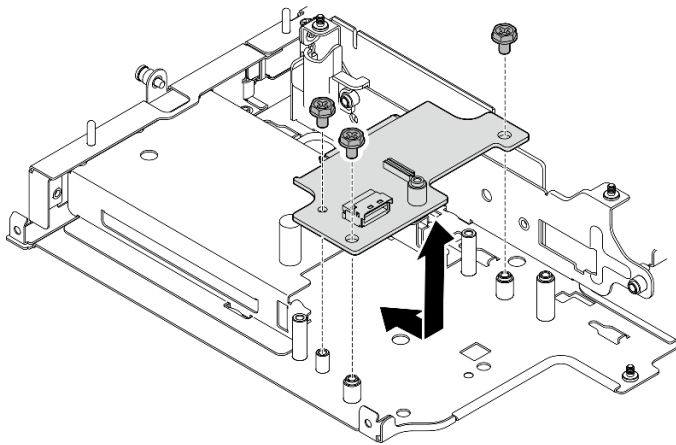
圖例 230. 卸下背板 1
