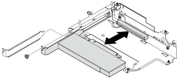
圖例 234. 卸下 PCIe 配接卡
