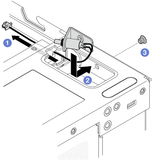
圖例 169. 安裝鎖定位置開關及纜線
