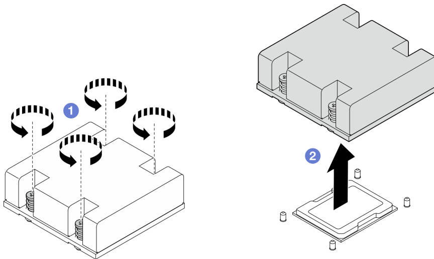
圖例 217. 卸下處理器散熱槽
