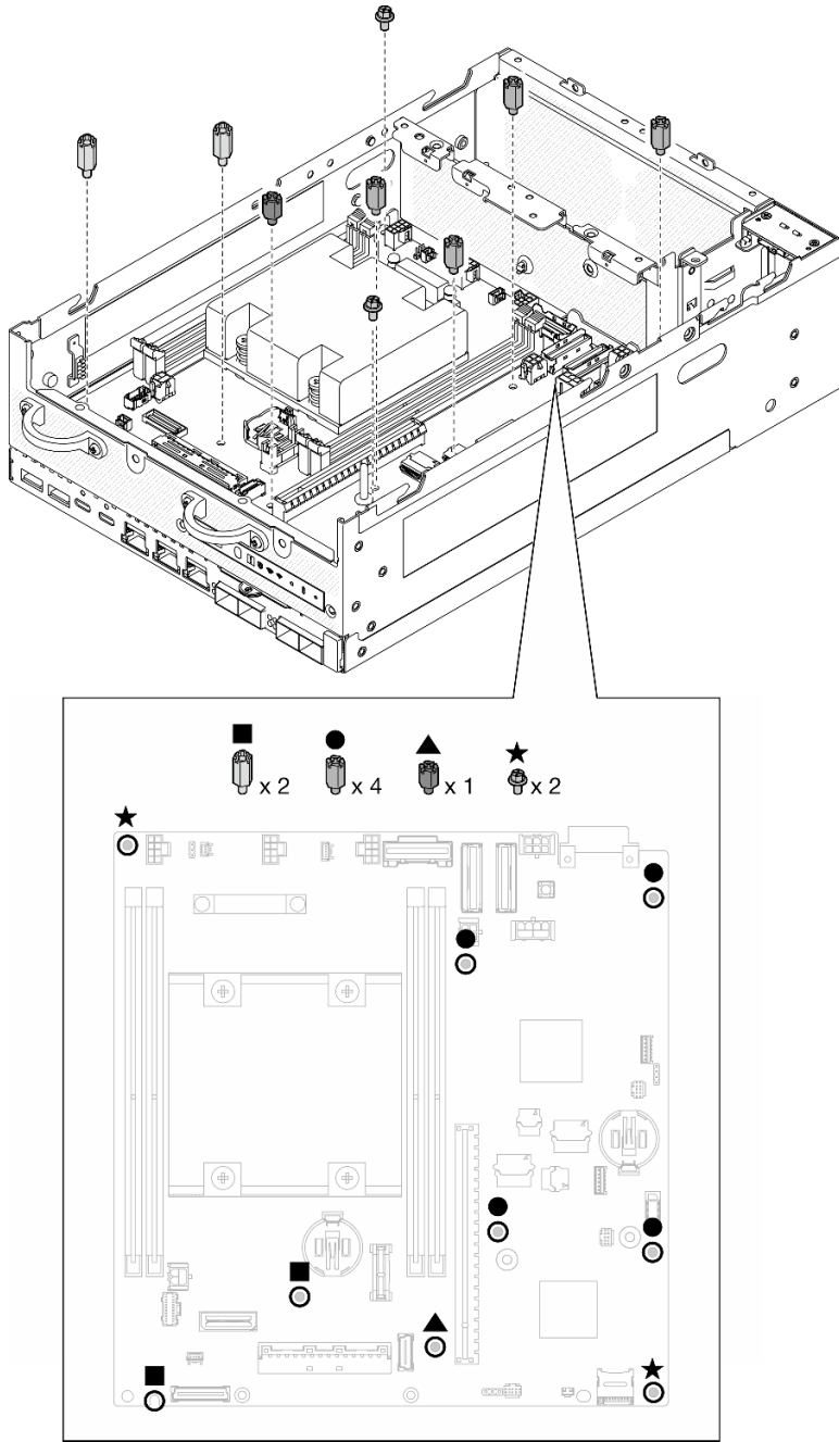
圖例 272. 主機板上的螺絲和支座
