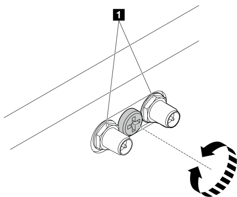
圖例 30. 縮短 SMA 接頭
