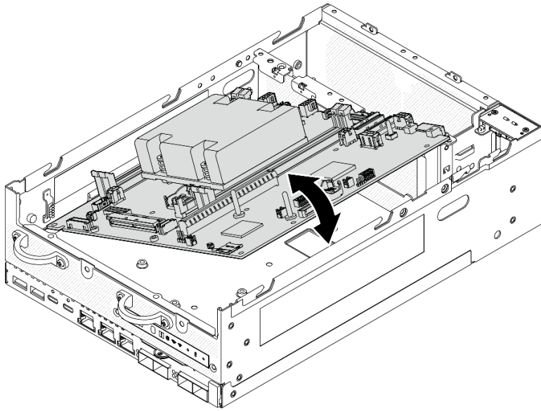
圖例 273. 卸下主機板
