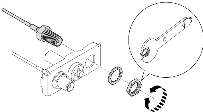
圖例 319. 從托架上鬆開纜線
