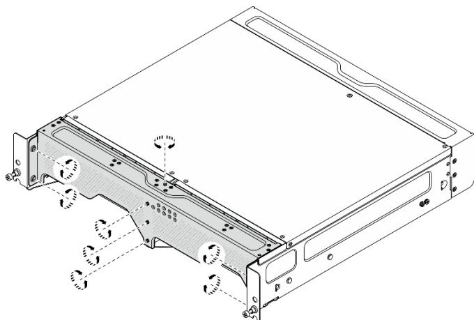
圖例 71. 鎖緊螺絲
