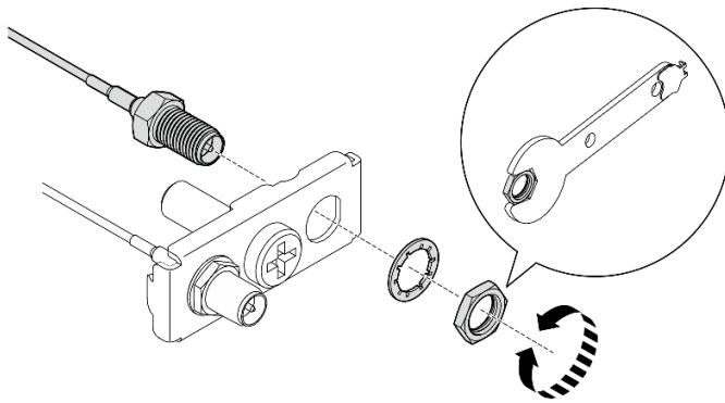
圖例 308. 從托架上鬆開纜線
