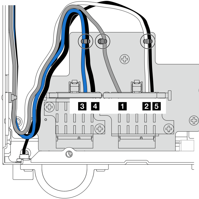
圖例 330. 無線配接卡的纜線佈線
