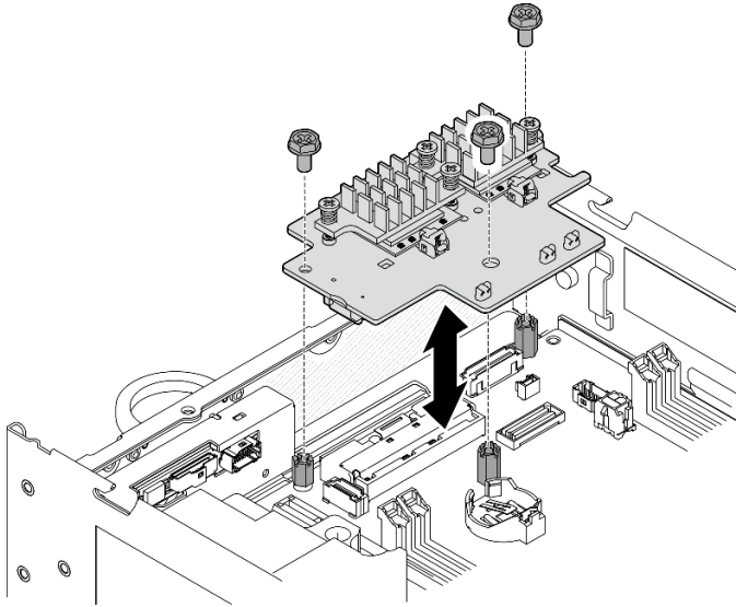
圖例 93. 提起無線配接卡
