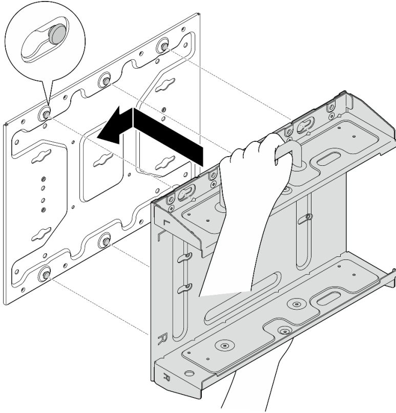
圖例 35. 組裝節點套筒
