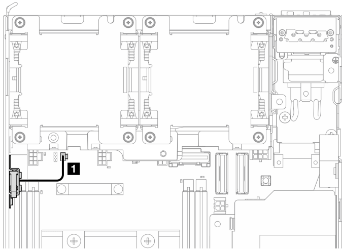
圖例 147. 頂部入侵開關纜線佈線
