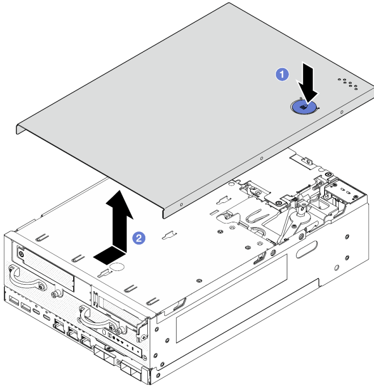
圖例 185. 卸下上蓋
