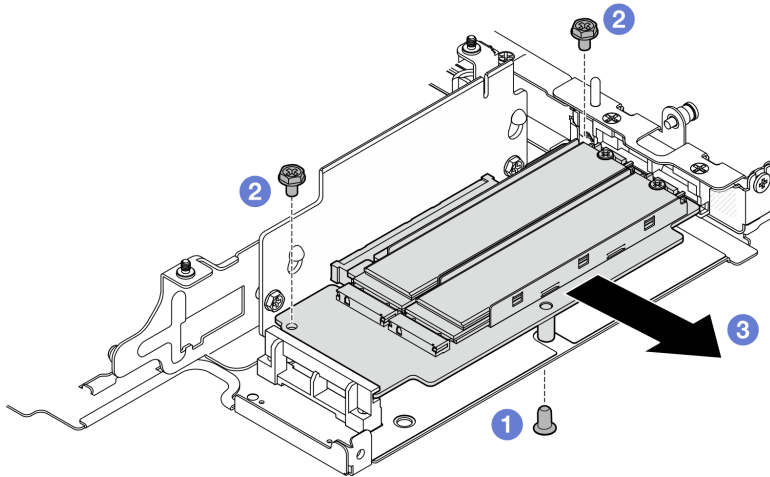
圖例 236. 卸下 M.2 配接卡
