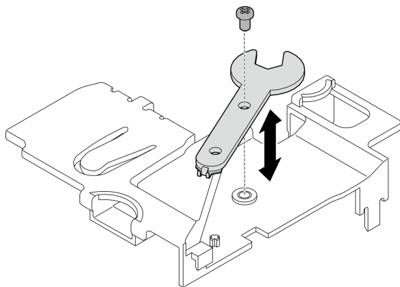
圖例 298. 鬆開扳手
