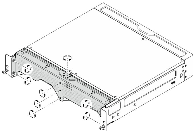
圖例 25. 鎖緊螺絲
