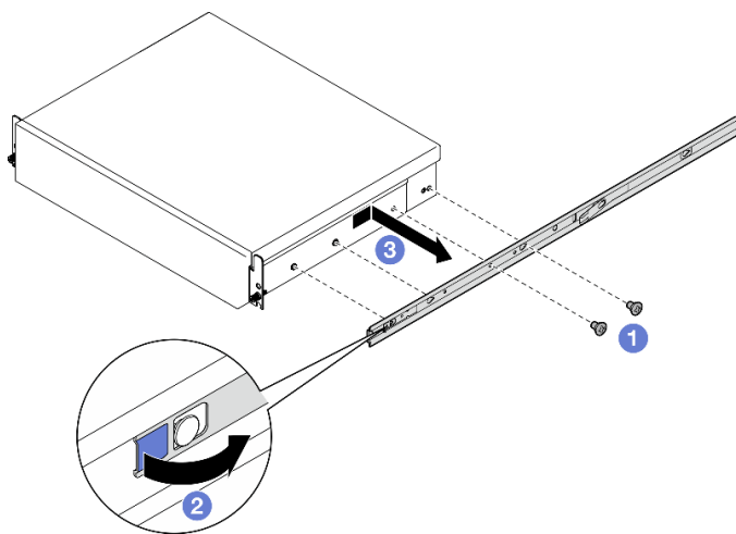
圖例 9. 卸下內滑軌
