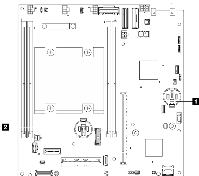
圖例 117. 主機板上的 CMOS 電池位置
