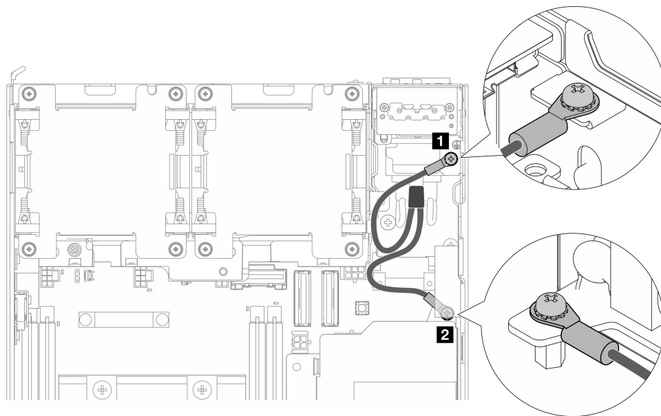
圖例 140. 連接接地纜線
