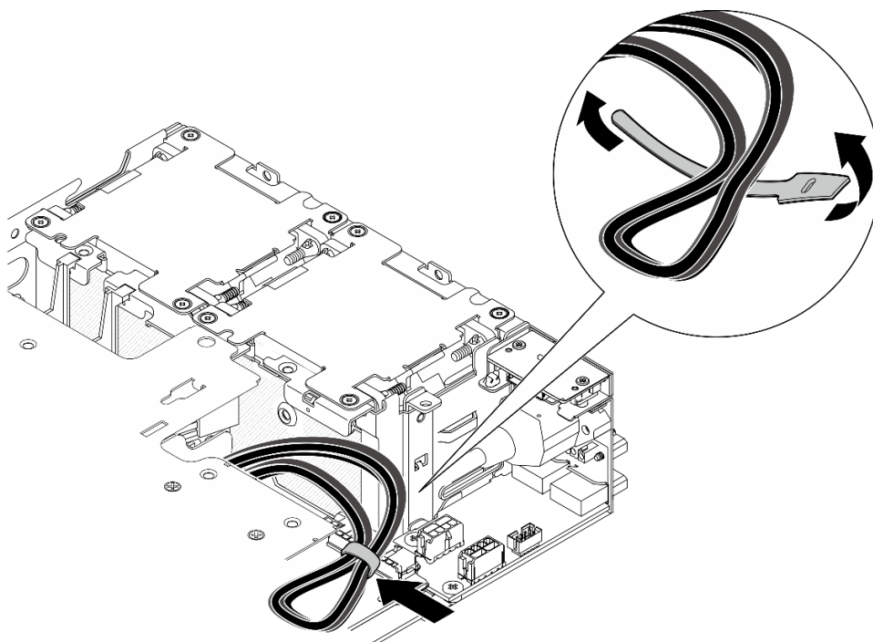
圖例 269. 擴充卡組件的纜線佈線
