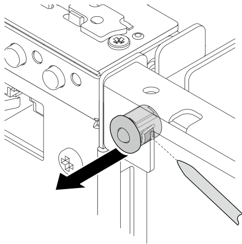
圖例 198. 卸下 PMB 狀態 LED 纜線
