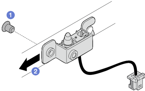
圖例 149. 卸下入侵開關及纜線
