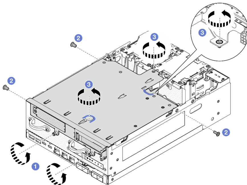
圖例 222. 鬆開擴充卡組件
