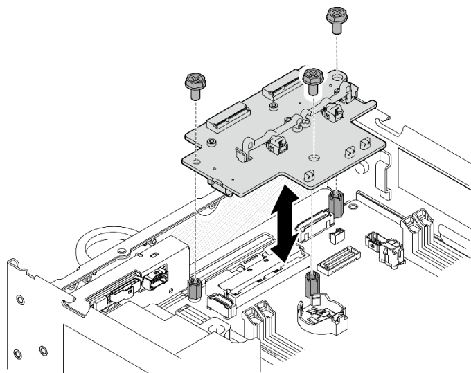
圖例 284. 安裝無線配接卡
