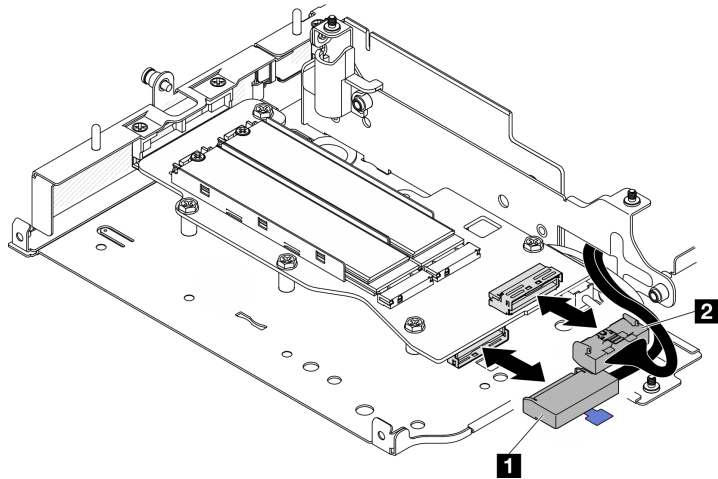
圖例 249. 拔掉信號線
