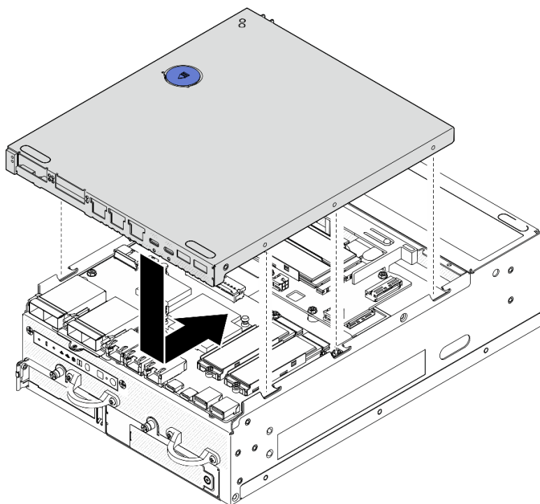
圖例 194. 安裝底蓋
