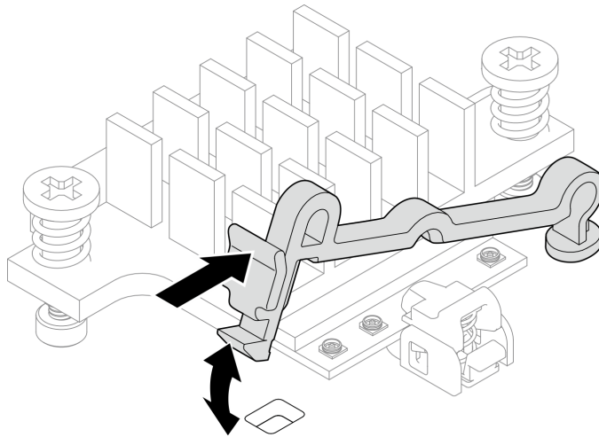
圖例 305. 插入纜線固定器
