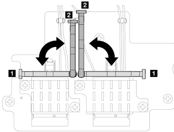
圖例 313. 轉動纜線固定器
