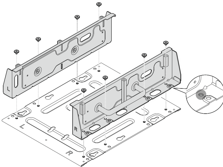
圖例 34. 組裝節點套筒
