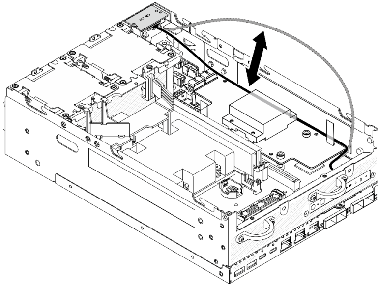
圖例 207. 放置信號線
