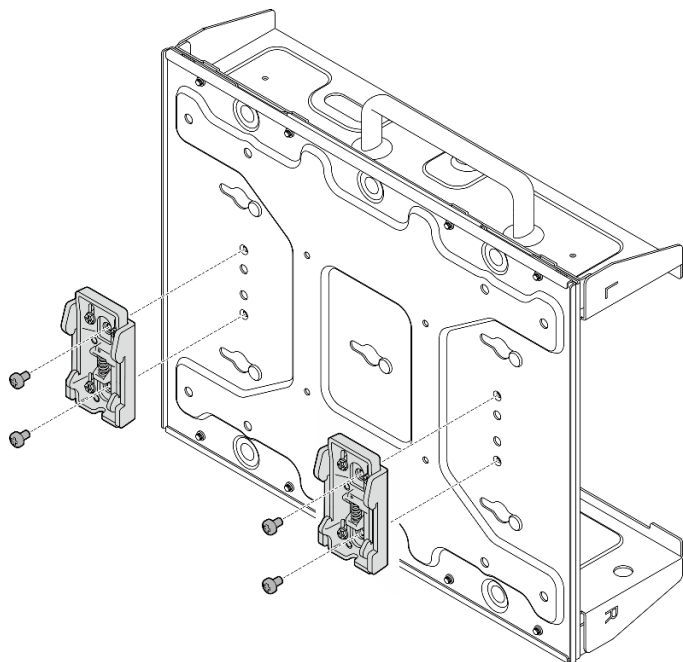
圖例 53. 卸下 DIN 滑軌固定夾
