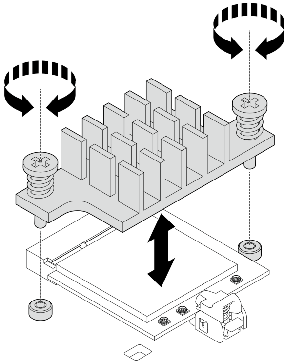
圖例 281. 卸下 WLAN/藍牙模組散熱槽
