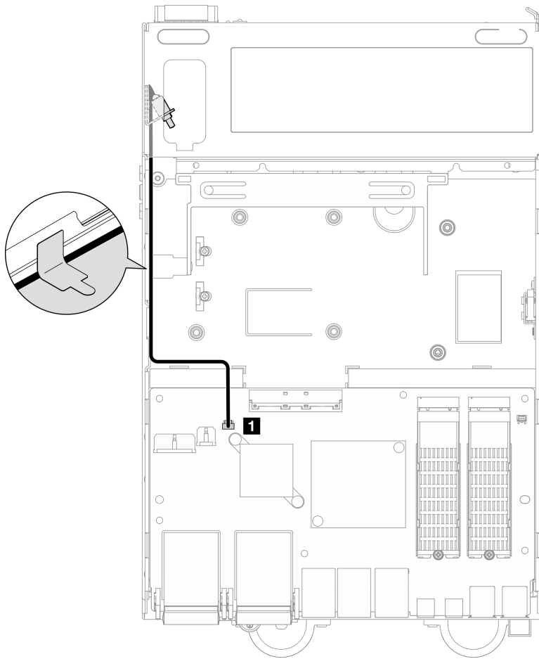
圖例 170. 鎖定位置開關纜線佈線
