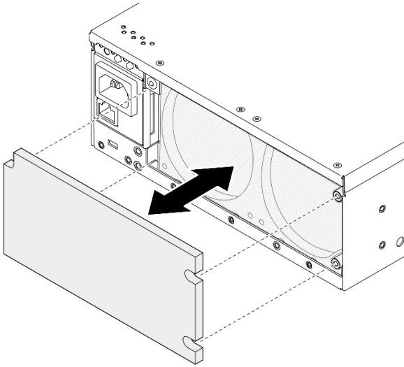
圖例 73. 卸下灰塵過濾器
