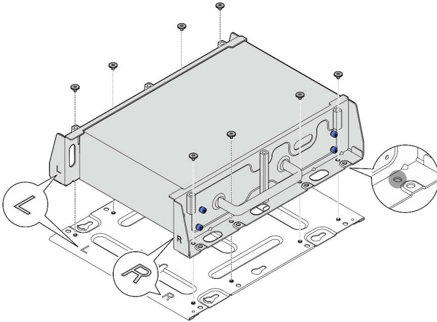
圖例 31. 卸下底板
