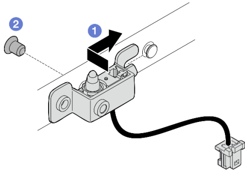
圖例 146. 安裝入侵開關及纜線
