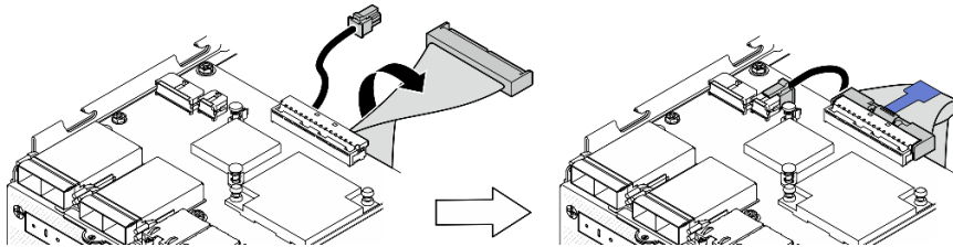
圖例 161. 連接 I/O 板纜線
