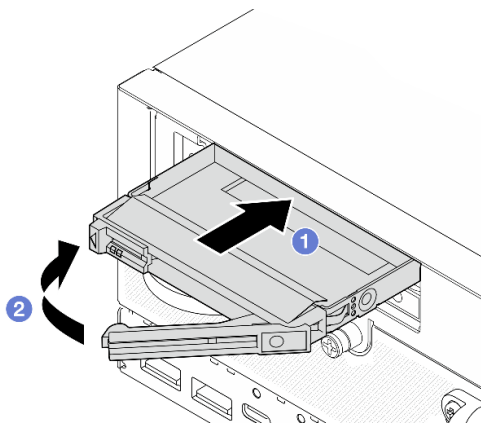
圖例 80. 安裝硬碟填充板
