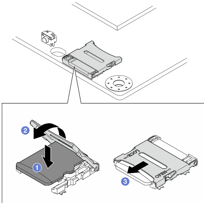
圖例 183. 安裝 MicroSD 卡
