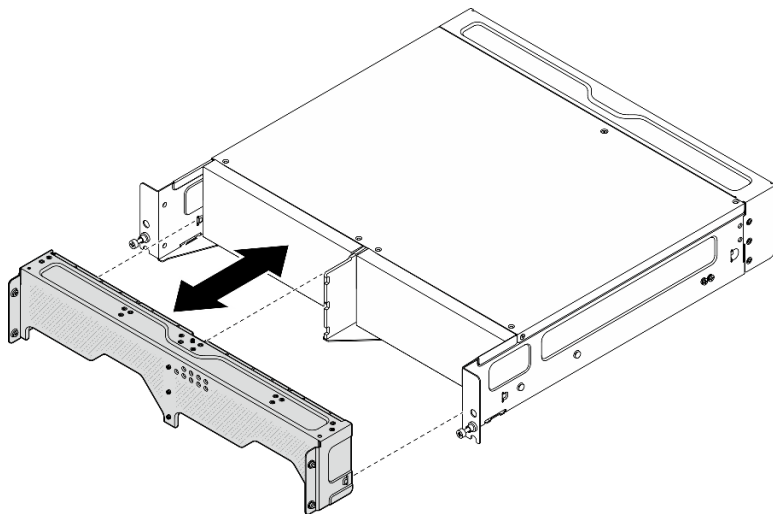
圖例 24. 安裝出貨托架
