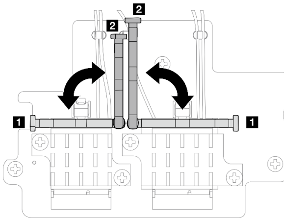
圖例 332. 轉動纜線固定器
