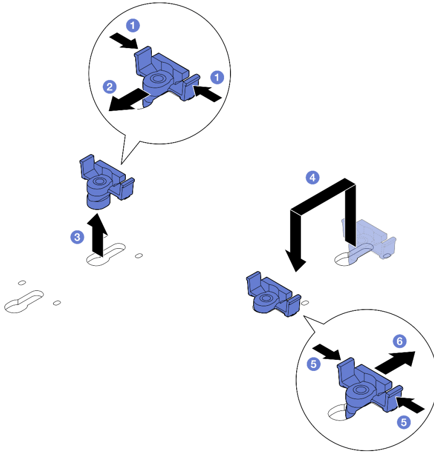
圖例 114. 調整 M.2 固定器
