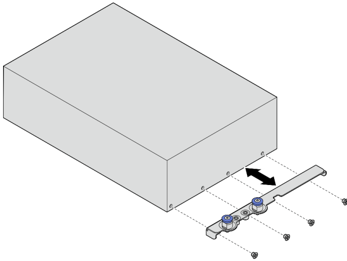
圖例 20. 安裝機體托架
