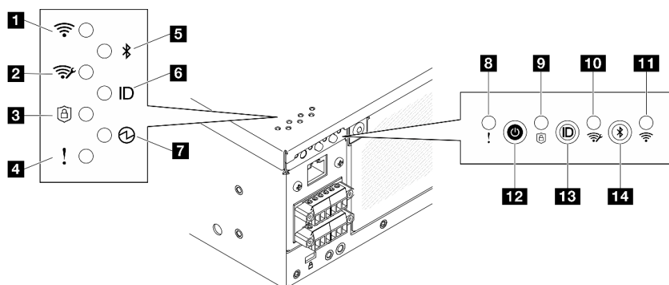
圖例 350. 後方操作面板 LED
