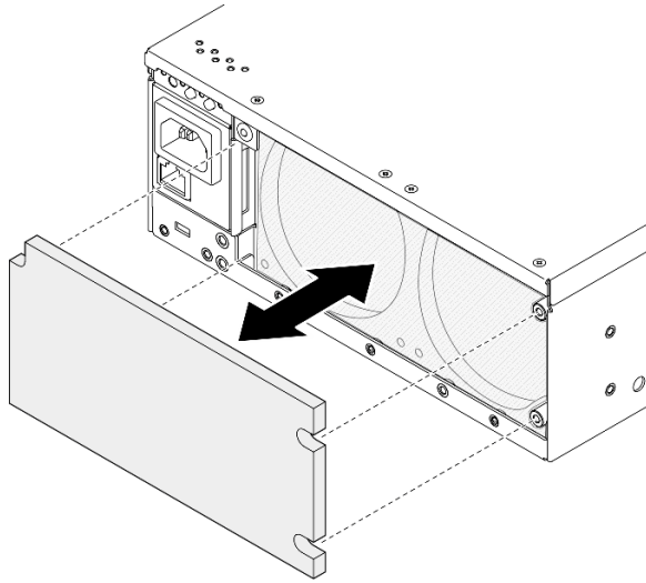
圖例 74. 安裝灰塵過濾器
