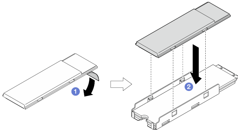
圖例 175. 安裝 M.2 散熱槽
