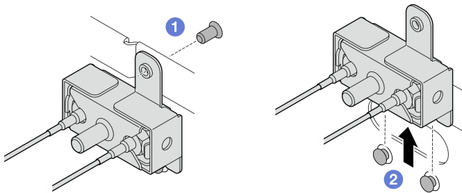
圖例 306. 卸下 SMA 組件
