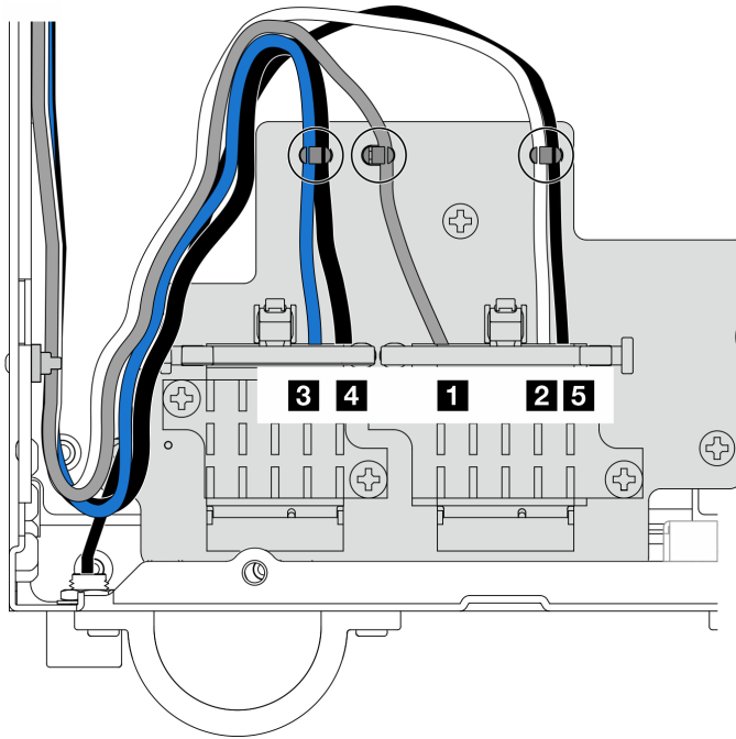
圖例 294. 無線配接卡的纜線佈線
