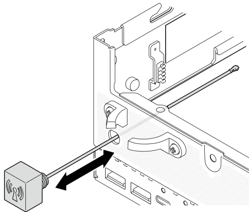
圖例 100. 卸下藍牙天線
