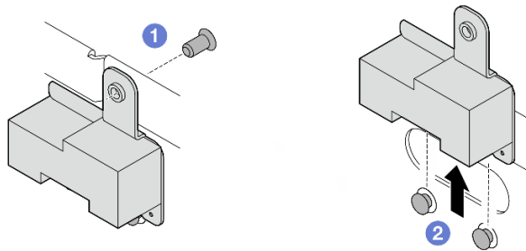
圖例 311. 卸下 SMA 填充板
