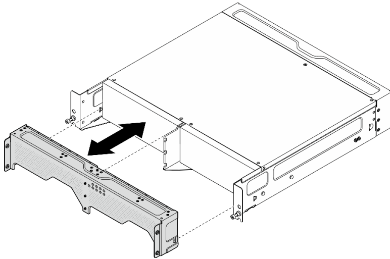
圖例 3. 卸下出貨托架
