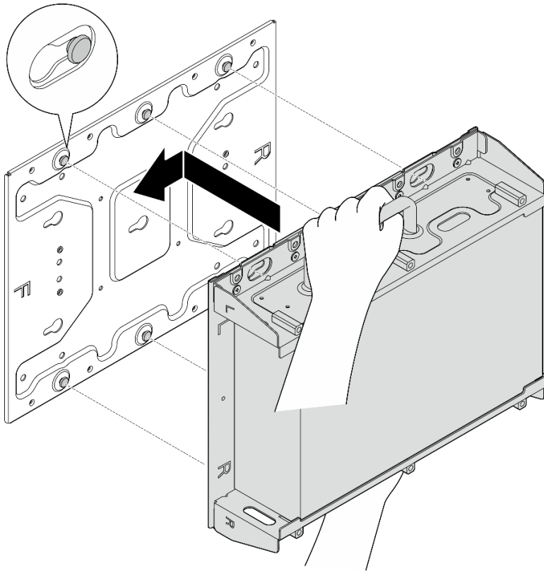
圖例 47. 安裝節點托架
