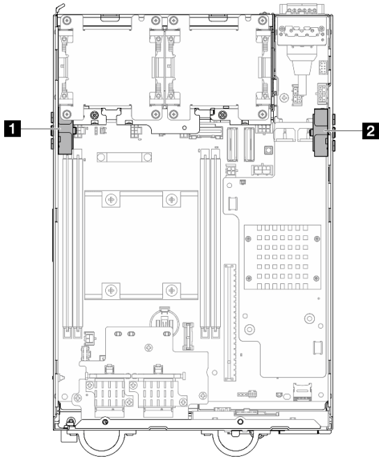
圖例 323. SMA 組件位置
