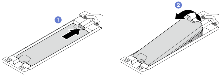
圖例 231. 卸下地理位置追蹤模組
