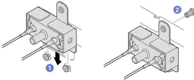
圖例 326. 安裝 SMA 組件
