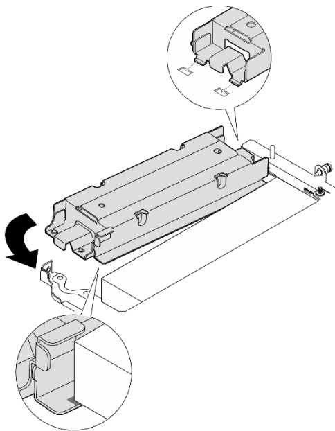
圖例 256. 安裝地理位置追蹤模組盒
