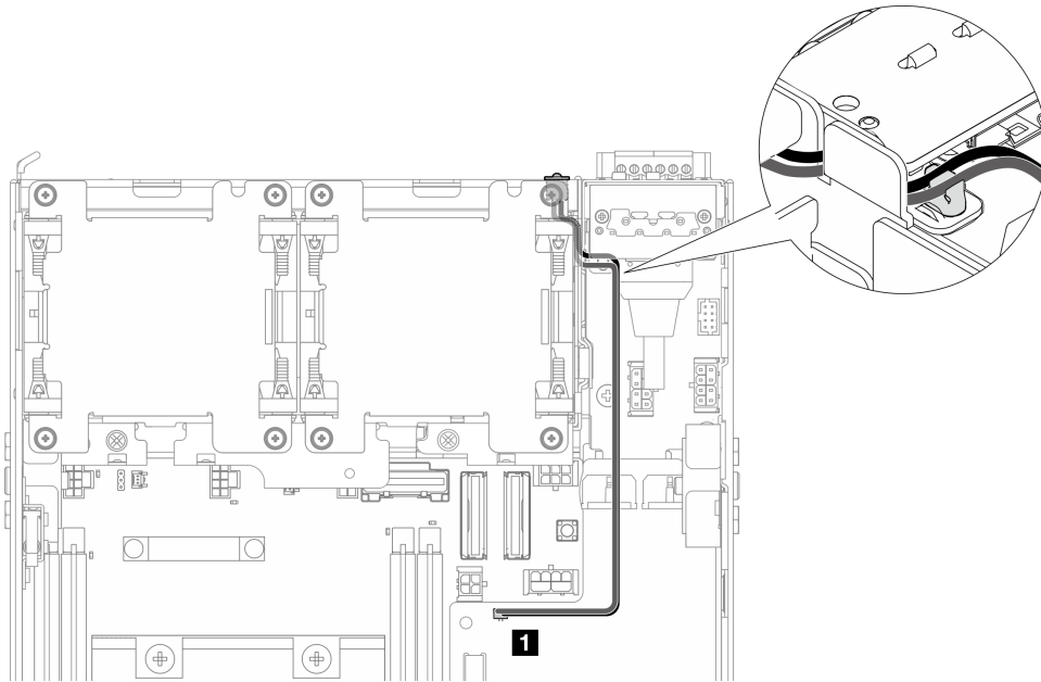
圖例 208. PMB LED 纜線
