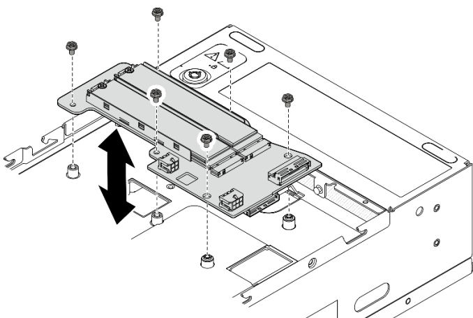
圖例 113. 卸下底部 M.2 含纜線配接卡
