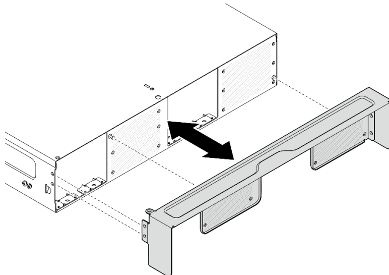
圖例 12. 安裝出貨托架
