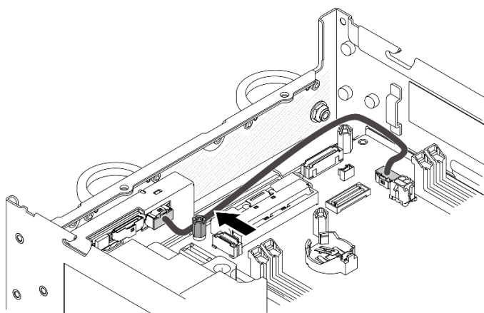
圖例 341. 前方操作面板纜線佈線
