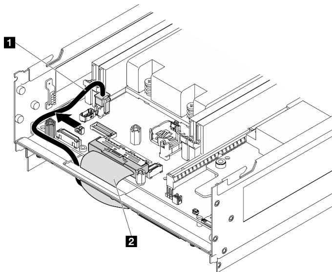
圖例 276. I/O 板纜線佈線
