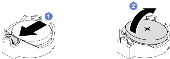
圖例 119. 取出 CMOS 電池
