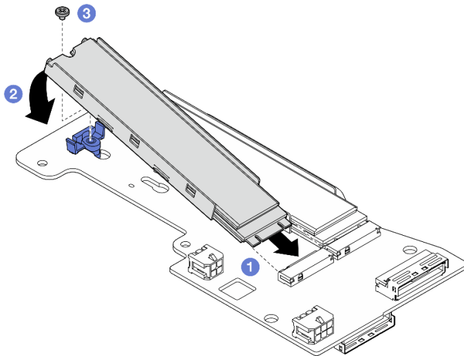
圖例 116. 安裝 M.2 硬碟
