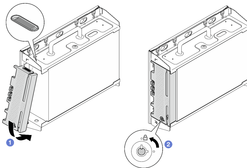
圖例 65. 安裝安全擋板
