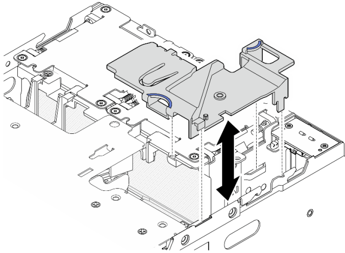
圖例 84. 卸下空氣擋板
