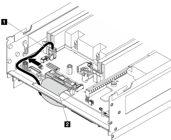
圖例 158. I/O 板纜線佈線
