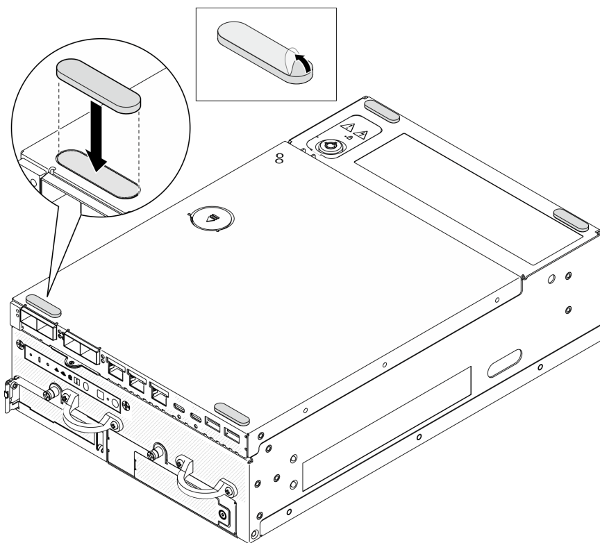
圖例 271. 安裝橡膠接腳
