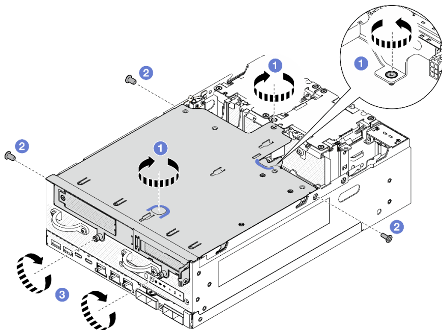
圖例 261. 固定擴充卡組件
