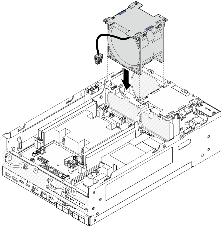
圖例 128. 安裝風扇模組
