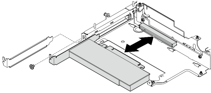
圖例 255. 安裝 PCIe 配接卡
