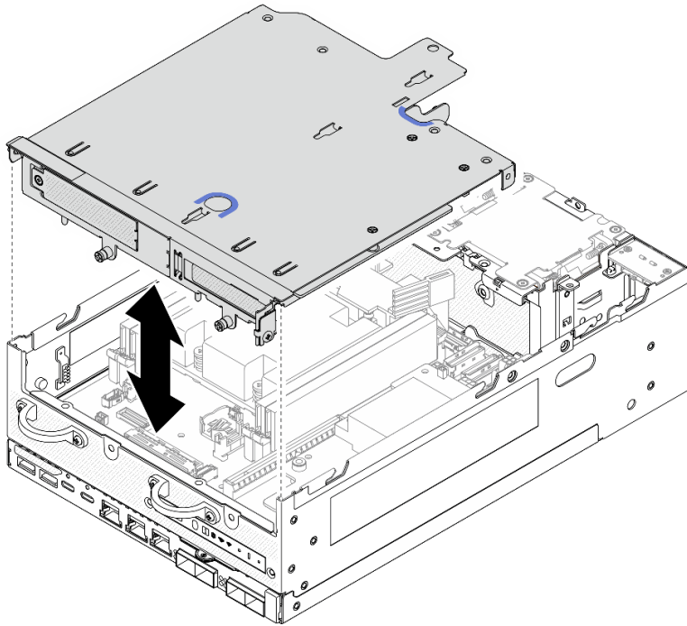
圖例 223. 抬起擴充卡組件
