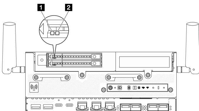
圖例 347. 硬碟 LED
