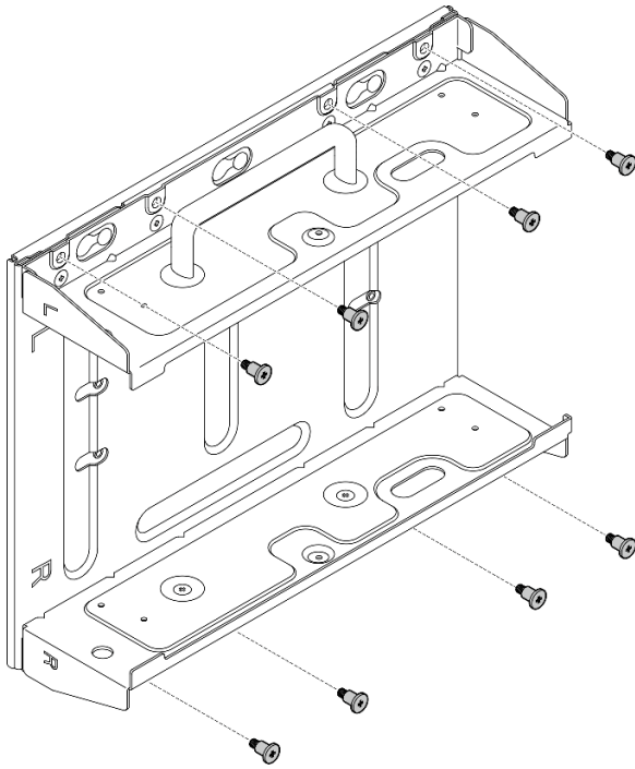
圖例 27. 卸下節點托架
