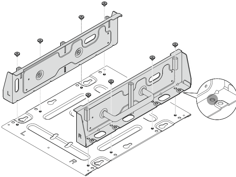
圖例 57. 組裝節點套筒
