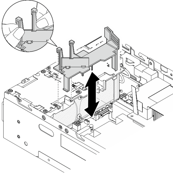
圖例 86. 卸下空氣擋板
