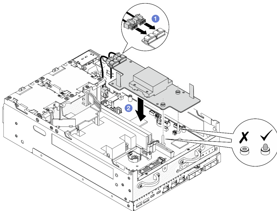
圖例 212. 安裝電源模組板
