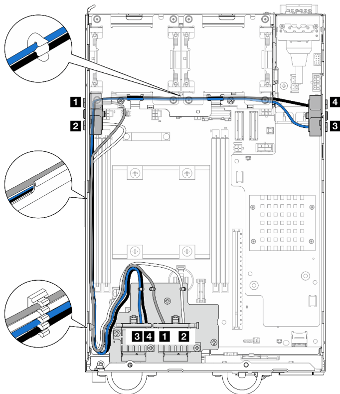
圖例 327. SMA 組件的纜線佈線
