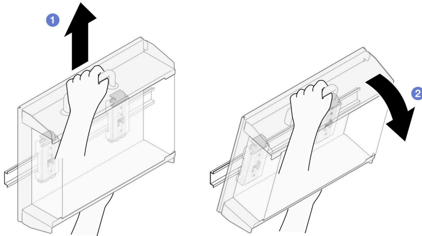
圖例 51. 卸下節點套筒
