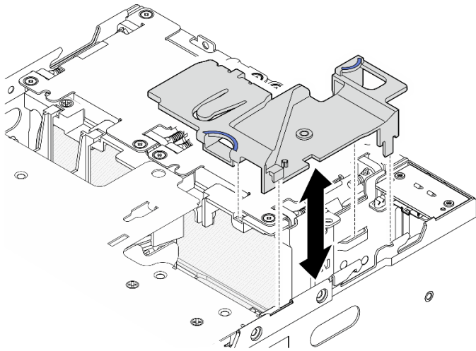
圖例 85. 安裝空氣擋板
