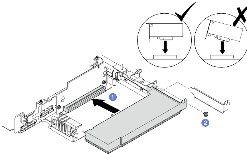
圖例 245. 安裝 PCIe 配接卡
