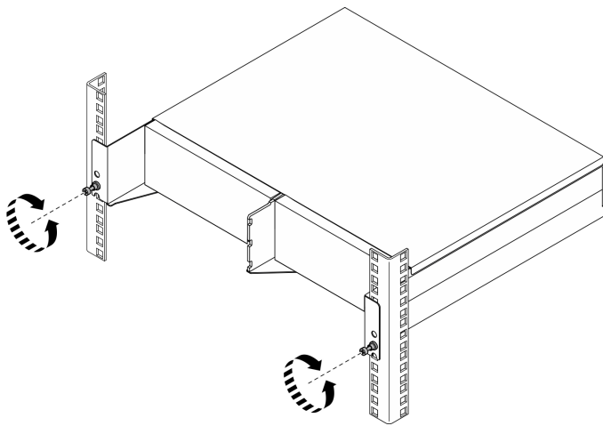
圖例 7. 使機體脫離機架
