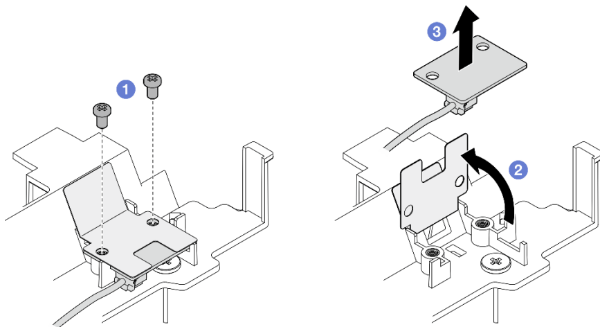
圖例 88. 卸下氣流感應器板
