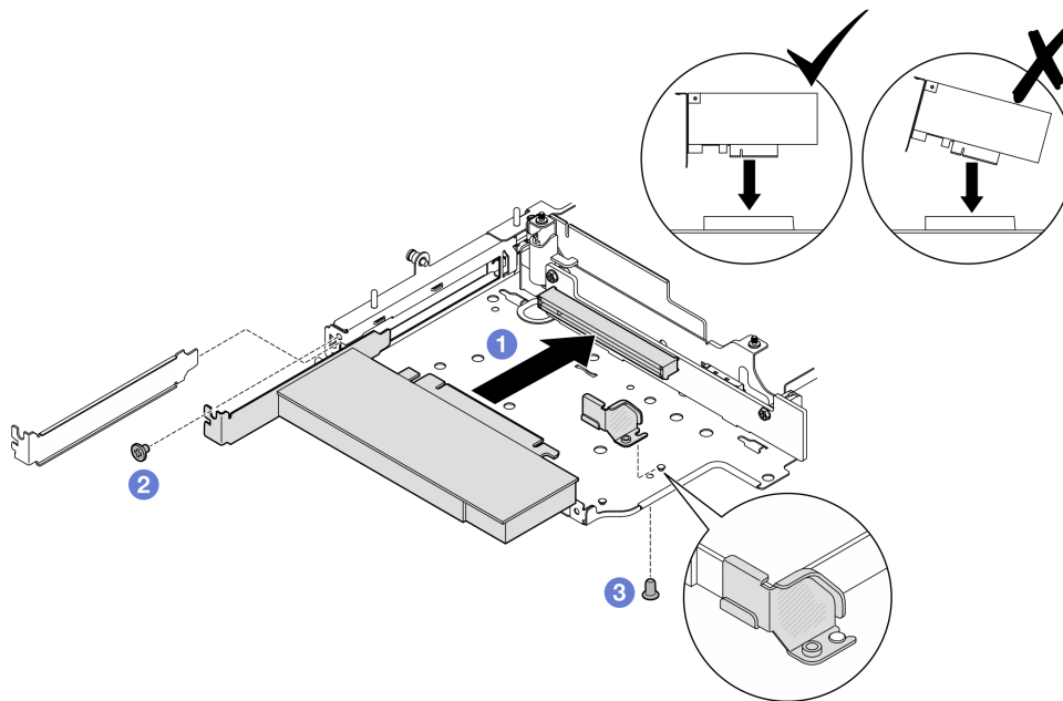
圖例 251. 安裝 PCIe 配接卡
