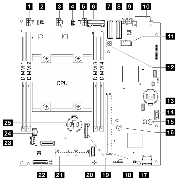
圖例 346. 主機板接頭
