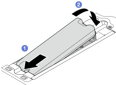
圖例 259. 安裝地理位置追蹤模組
