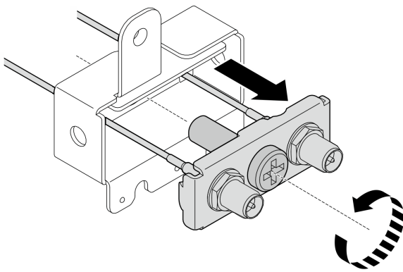
圖例 318. 卸下托架
