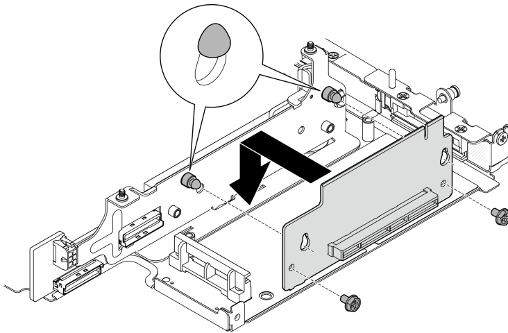
圖例 242. 安裝擴充卡
