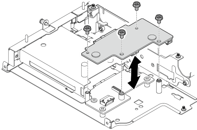
圖例 229. 卸下背板 2
