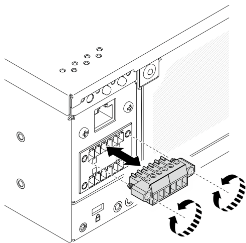
圖例 339. 安裝接頭
