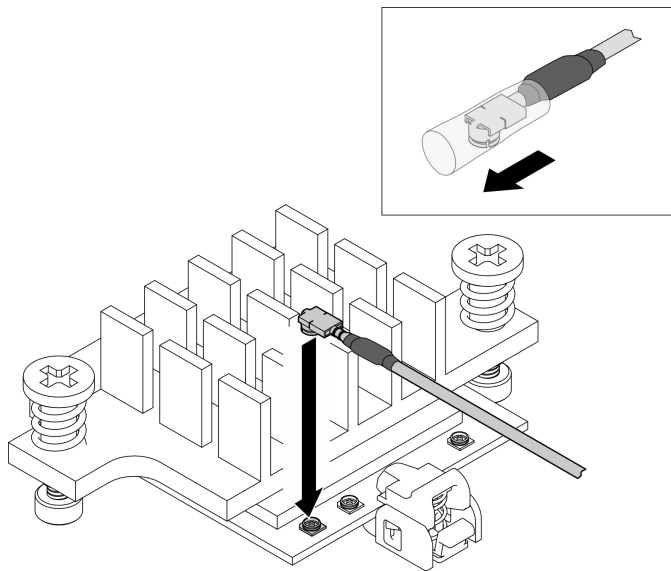
圖例 107. 連接纜線
