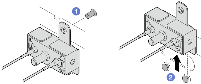
圖例 317. 卸下 SMA 組件
