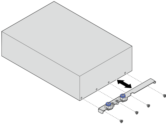
圖例 6. 卸下機體托架
