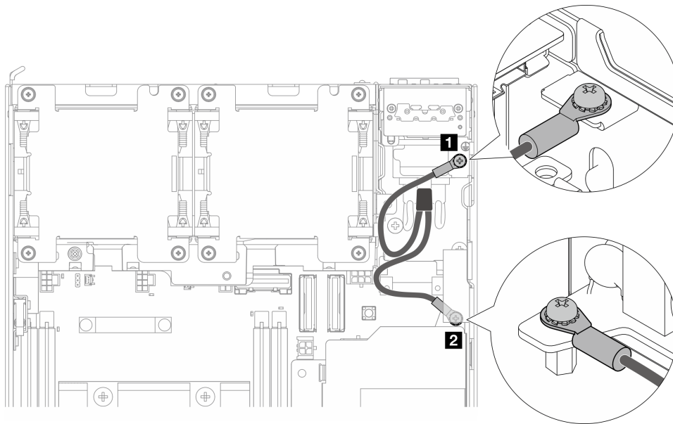
圖例 133. 拔下接地纜線
