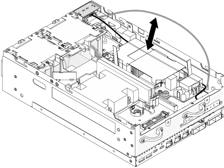
圖例 132. 放置信號線
