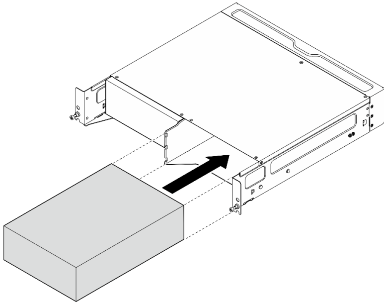
圖例 22. 安裝節點
