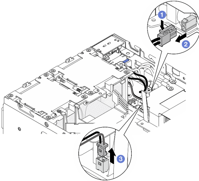
圖例 134. 拔下纜線
