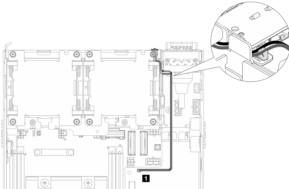
圖例 215. PMB LED 纜線
