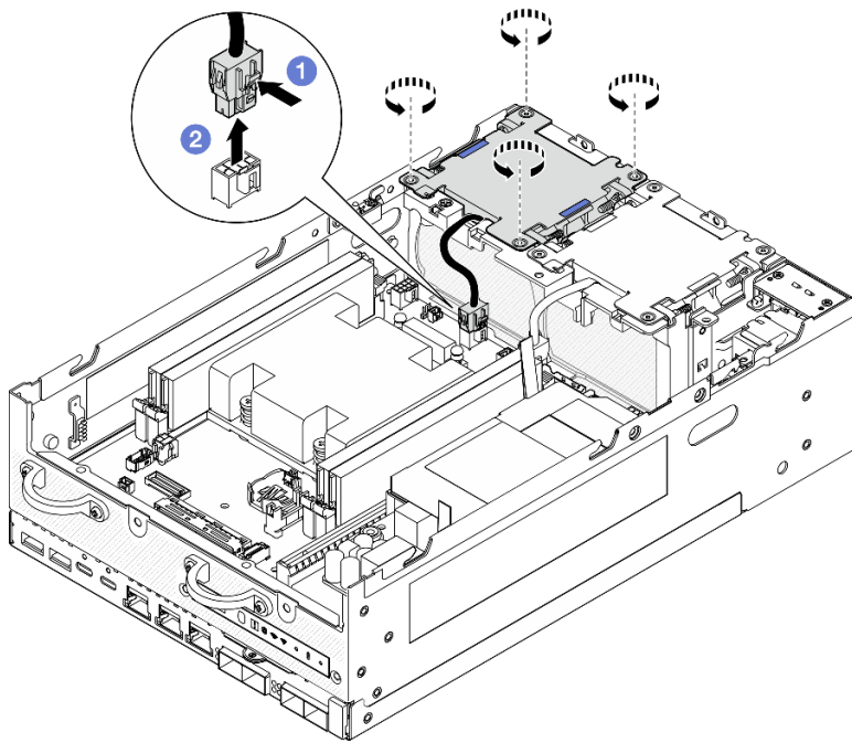
圖例 126. 卸下風扇模組
