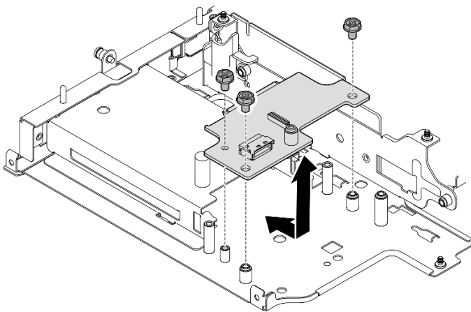
圖例 252. 安裝背板 1
