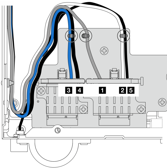
圖例 343. WLAN 天線和藍牙天線纜線佈線
