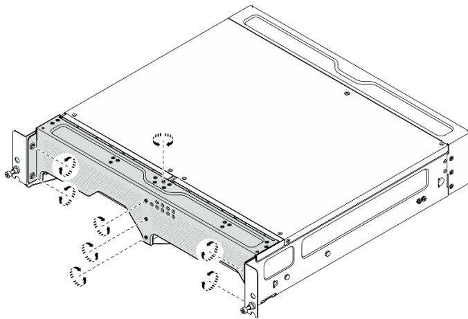
圖例 2. 鬆開螺絲
