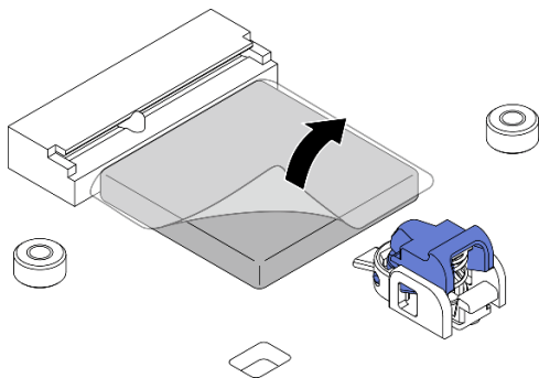
圖例 286. 取下散熱墊上的薄膜
