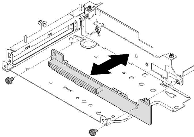
圖例 250. 安裝擴充卡
