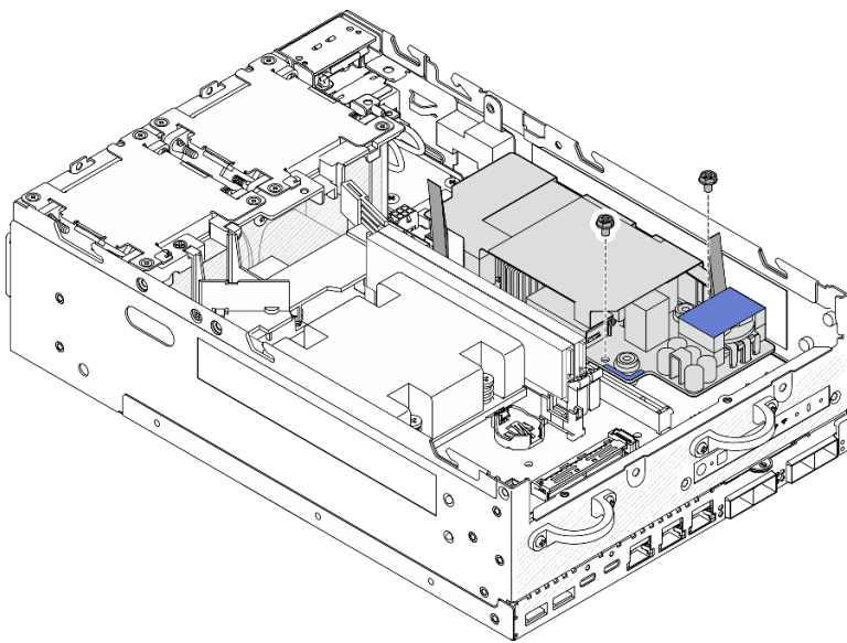
圖例 135. 鬆開螺絲
