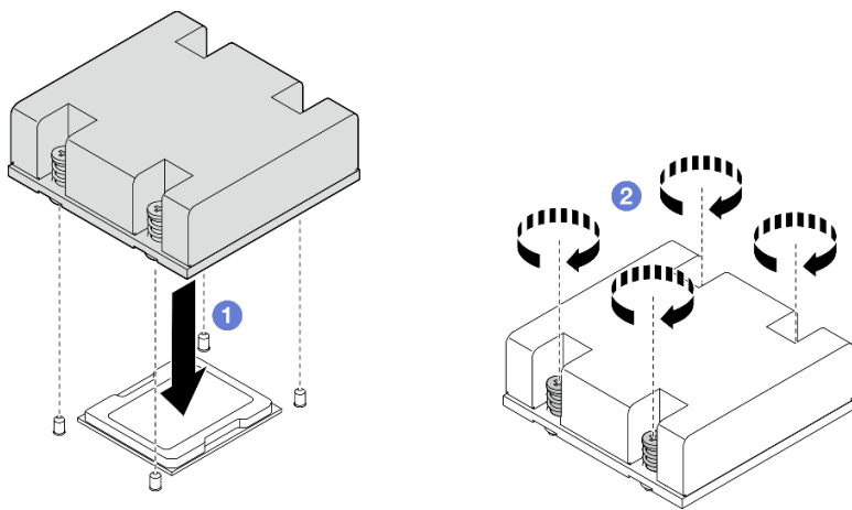
圖例 219. 安裝處理器散熱槽
