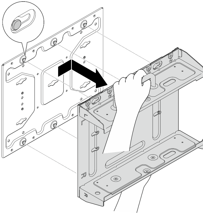
圖例 28. 卸下節點托架
