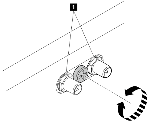
圖例 299. 縮短 SMA 接頭
