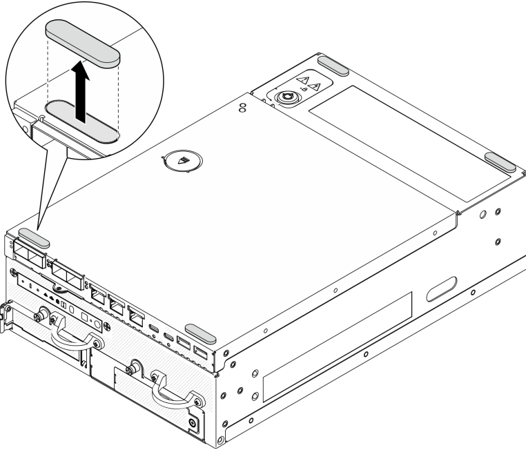
圖例 270. 卸下橡膠接腳
