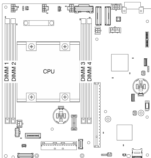
圖例 1. 記憶體模組和處理器佈置
