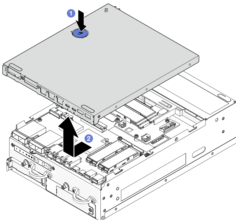
圖例 191. 卸下底蓋
