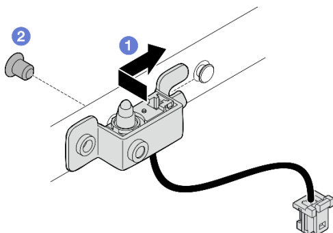
圖例 152. 安裝入侵開關及纜線
