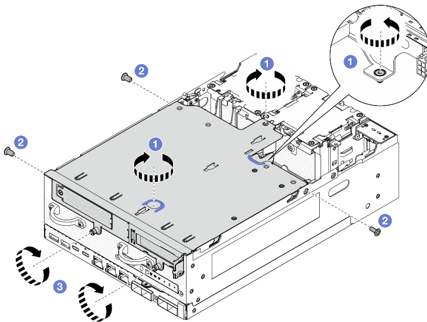
圖例 265. 固定擴充卡組件
