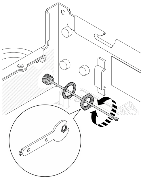
圖例 104. 安裝藍牙天線
