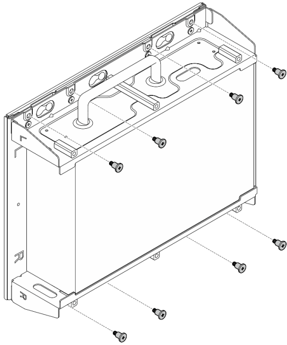
圖例 48. 安裝節點托架
