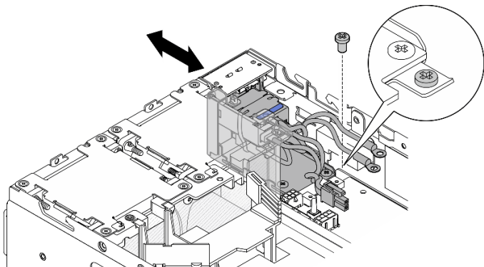
圖例 203. 卸下 AC PIB 模組
