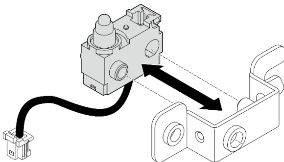
圖例 144. 將入侵開關與托架分開
