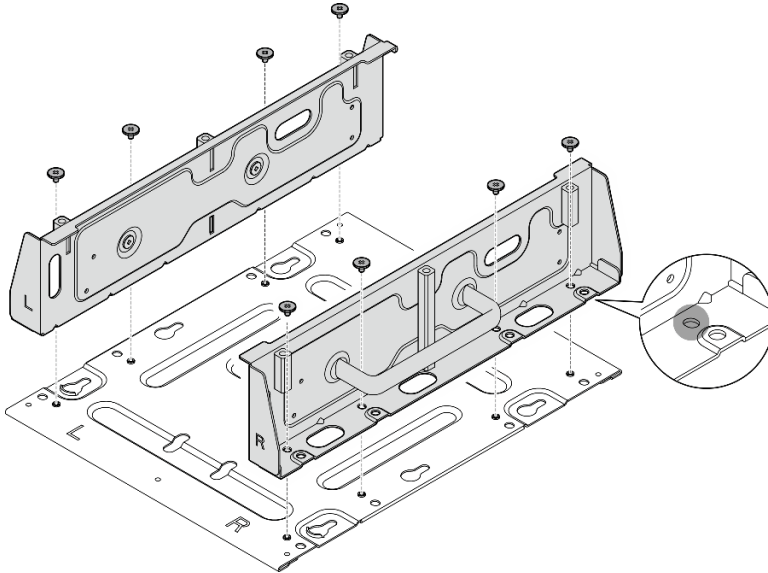
圖例 38. 拆卸節點托架
