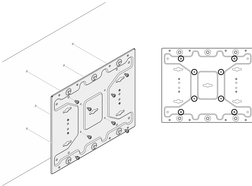
圖例 44. 安裝壁掛板
