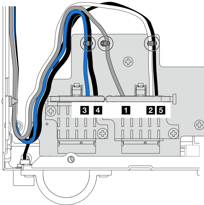
圖例 290. 無線配接卡的纜線佈線
