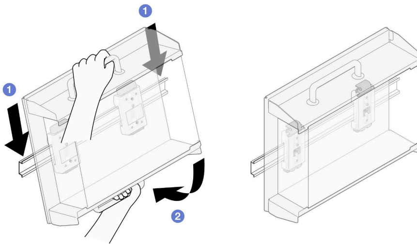
圖例 64. 安裝節點套筒
