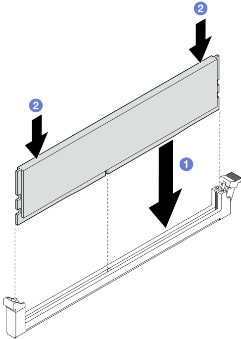
圖例 181. 安裝記憶體模組
