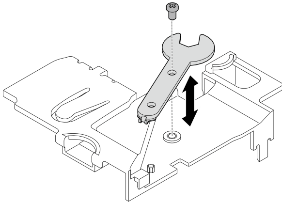
圖例 309. 存放扳手
