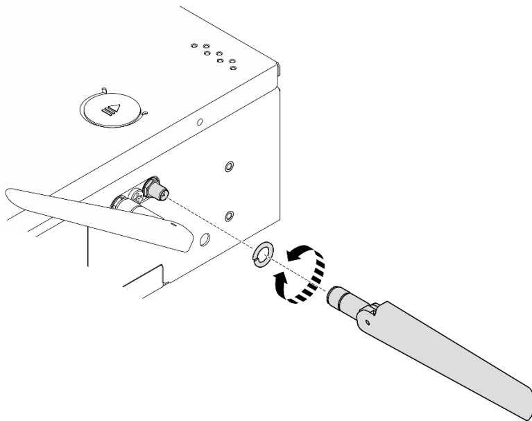
圖例 338. 安裝 WLAN 天線
