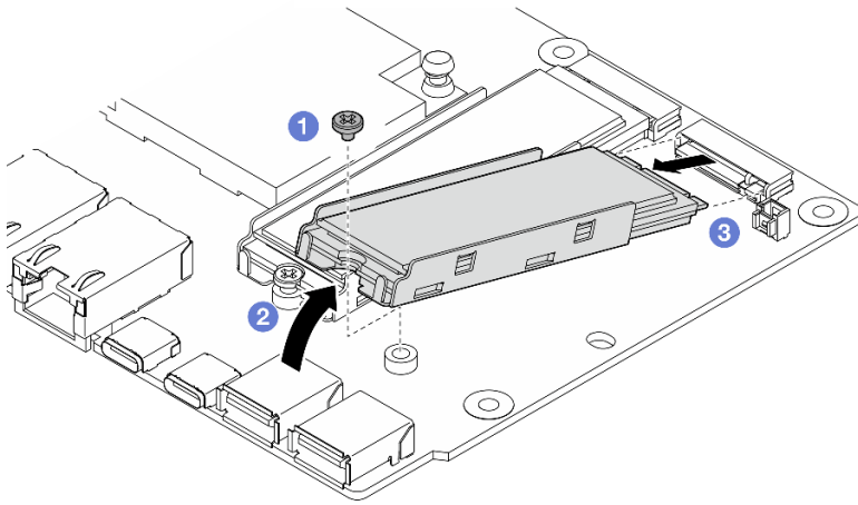
圖例 154. 卸下 M.2 硬碟
