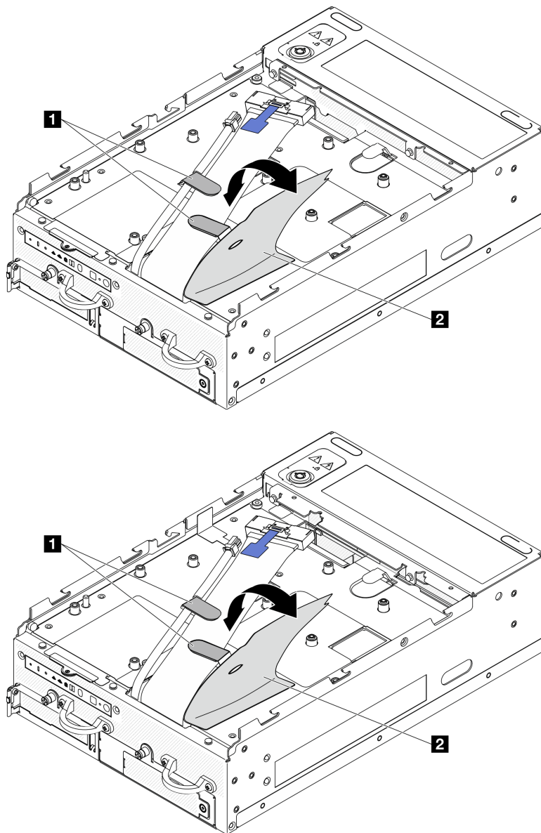
圖例 156. I/O 板纜線佈線
