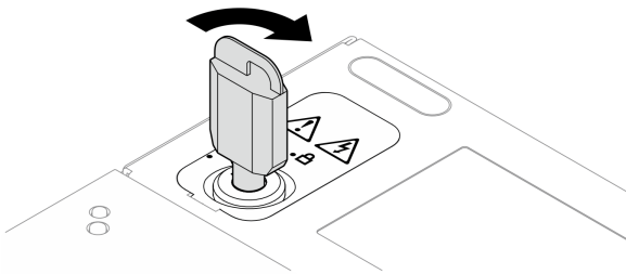
圖例 186. 鎖定鑰匙鎖
