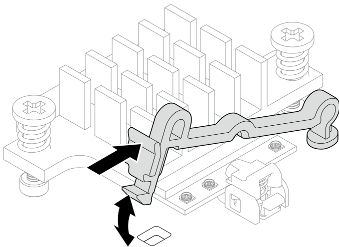
圖例 105. 提起纜線固定器
