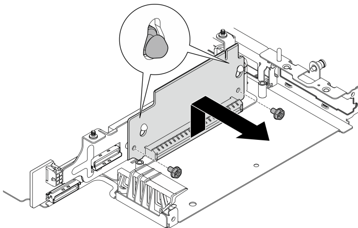
圖例 240. 卸下擴充卡
