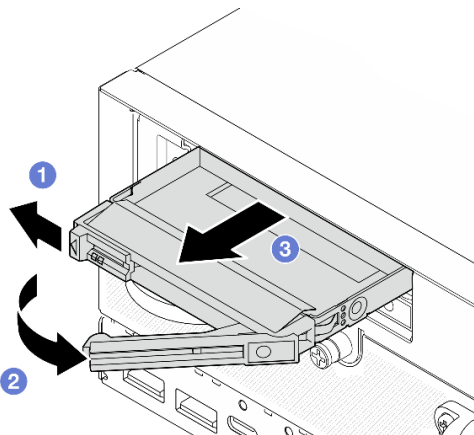
圖例 78. 卸下硬碟填充板
