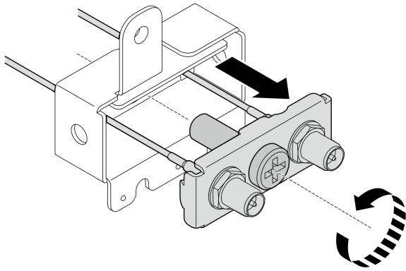
圖例 307. 卸下托架
