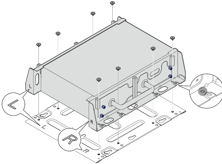
圖例 42. 安裝底板
