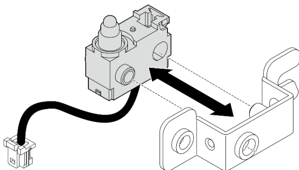
圖例 145. 將入侵開關插入托架
