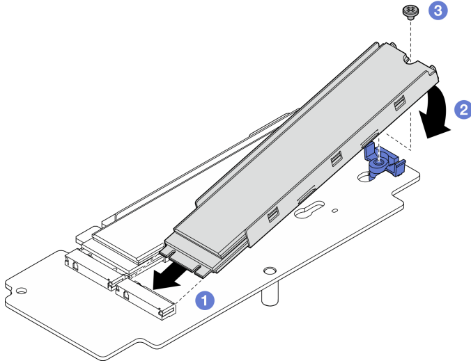
圖例 241. 安裝 M.2 硬碟
