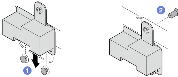
圖例 321. 安裝 SMA 填充板
