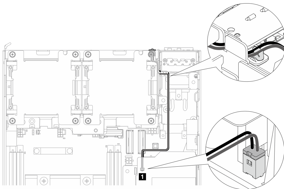
圖例 201. 連接到內部電源供應器 (AC PMB) 的 PMB 狀態 LED 纜線
