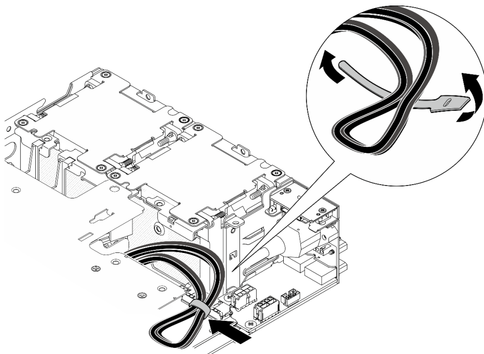
圖例 262. 擴充卡組件的纜線佈線
