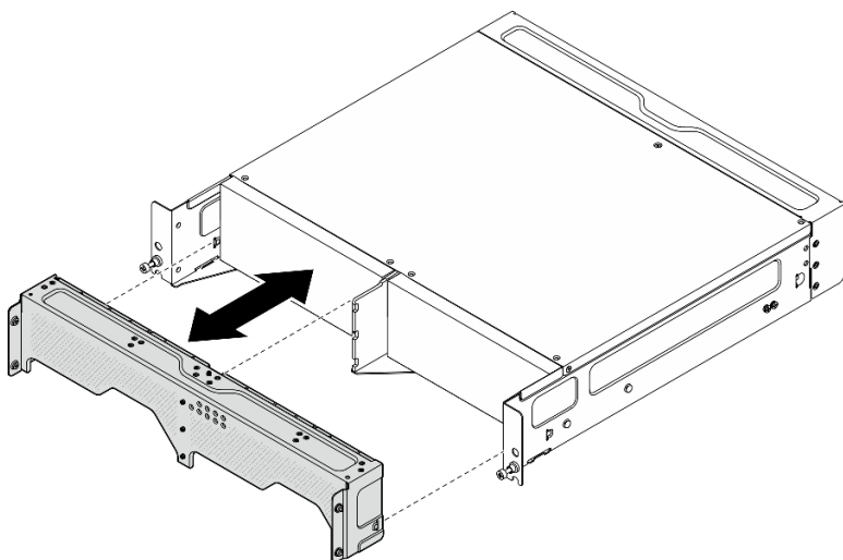
圖例 67. 卸下出貨托架
