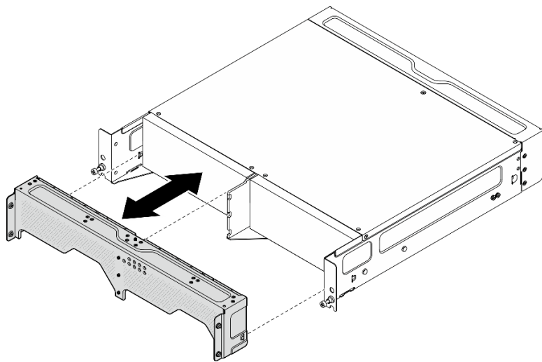
圖例 70. 安裝出貨托架
