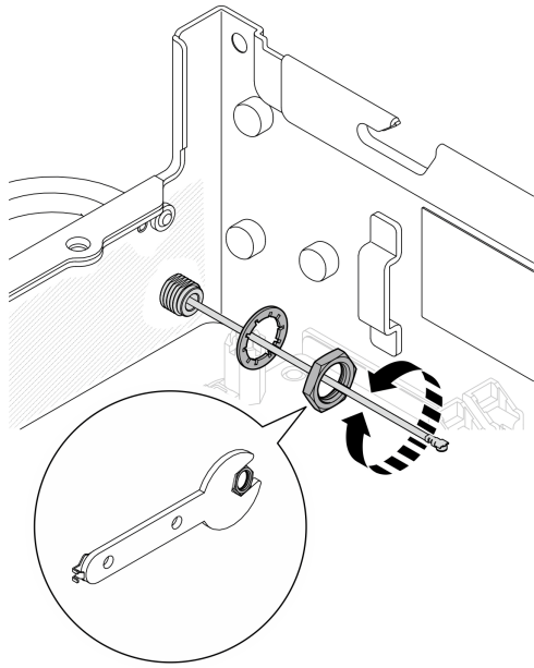
圖例 99. 卸下藍牙天線
