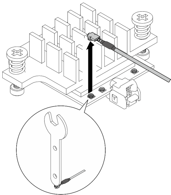
圖例 96. 拔下纜線
