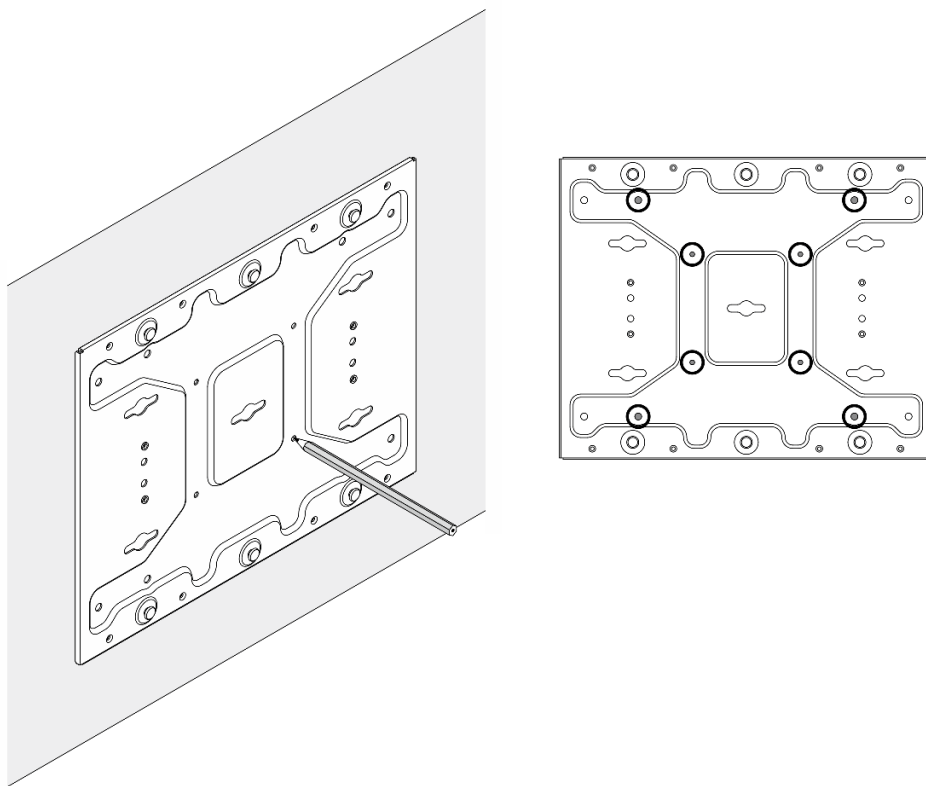
圖例 43. 螺絲孔的位置
