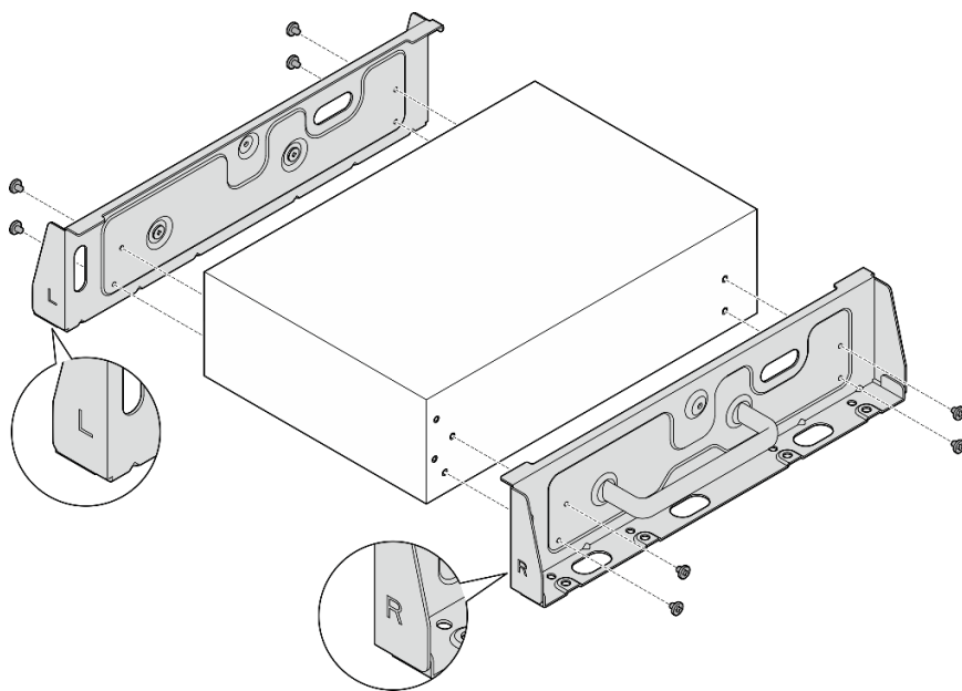
圖例 40. 用螺絲安裝側托架
