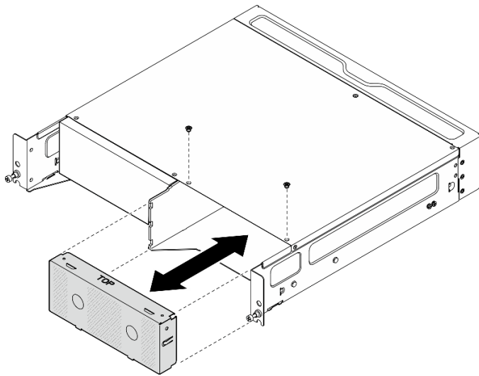
圖例 23. 安裝節點填充板
