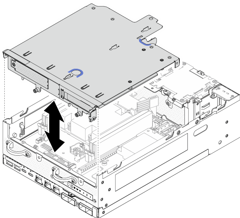
圖例 263. 放下擴充卡組件
