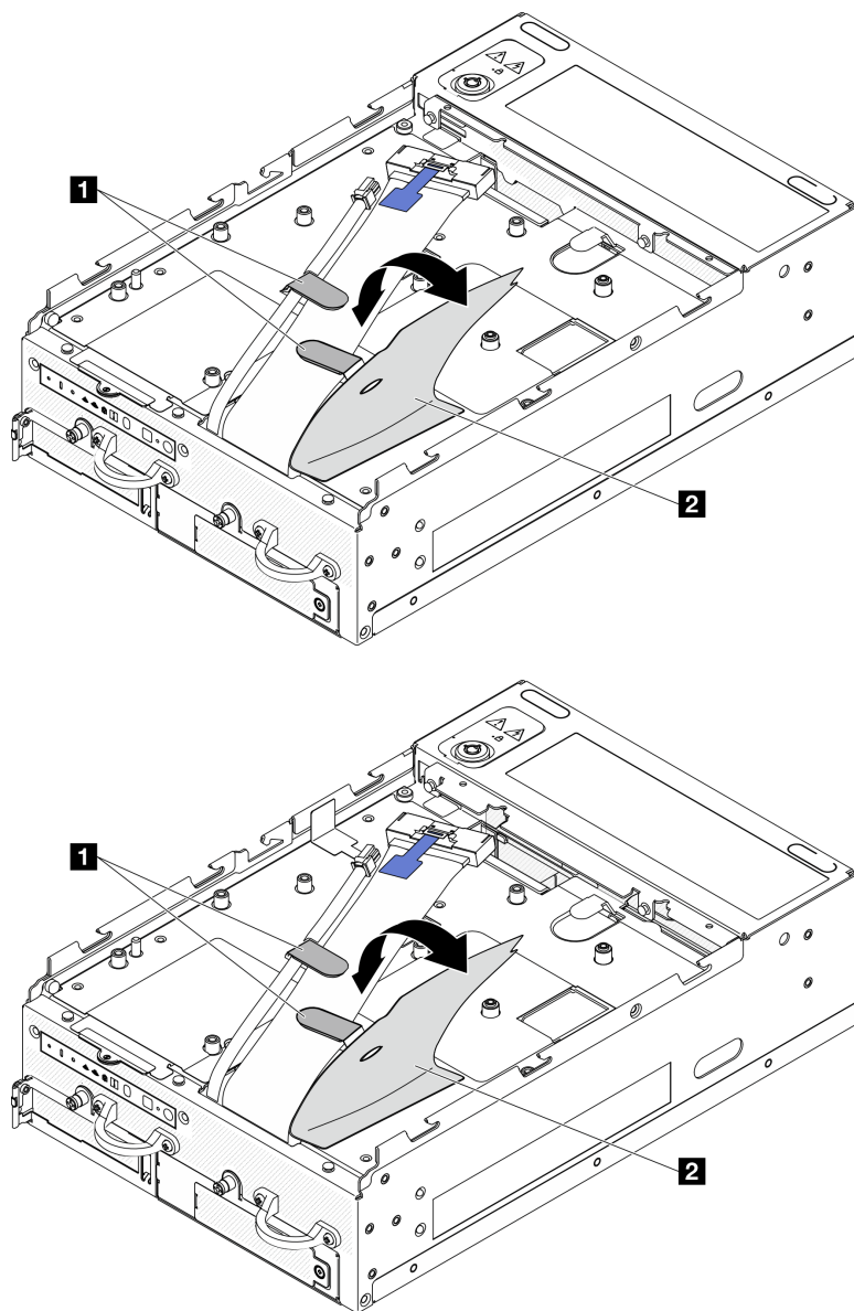
圖例 159. I/O 板纜線佈線
