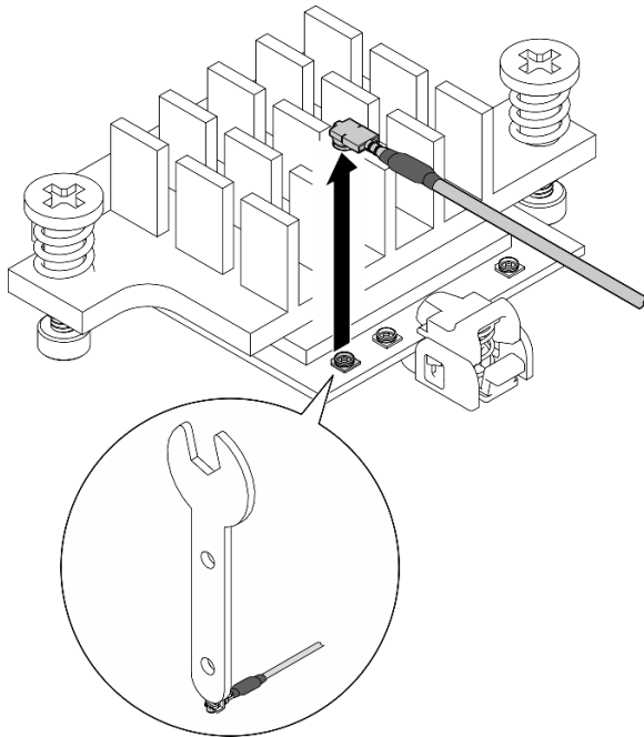
圖例 303. 拔下纜線
