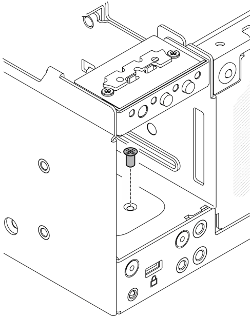
圖例 165. 鬆開螺絲
