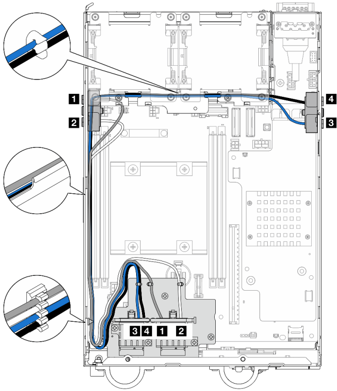
圖例 342. WLAN 天線纜線佈線
