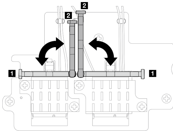
圖例 95. 轉動纜線固定器
