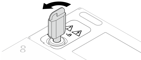
圖例 190. 解鎖鑰匙鎖
