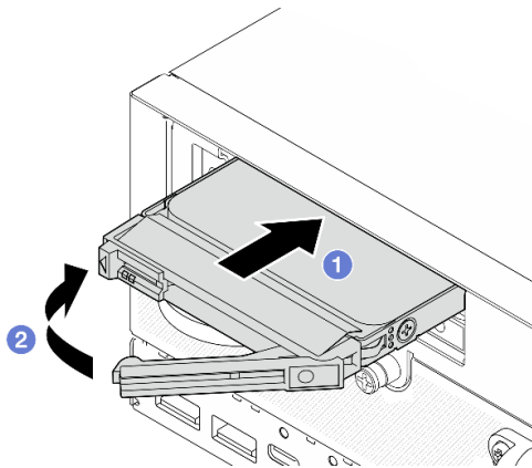
圖例 79. 安裝 7 公釐硬碟
