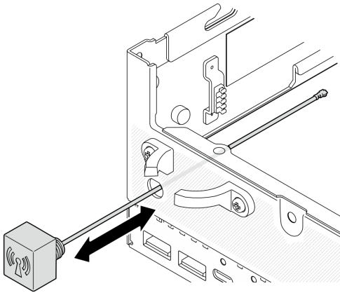
圖例 103. 安裝藍牙天線
