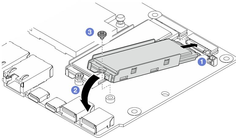
圖例 162. 安裝 M.2 硬碟
