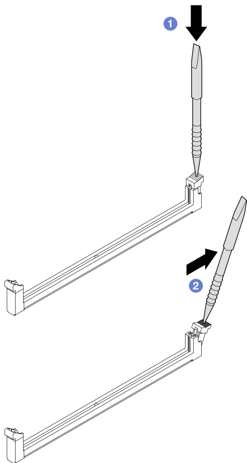
圖例 177. 打開固定夾
