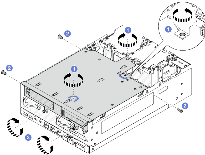
圖例 268. 固定擴充卡組件
