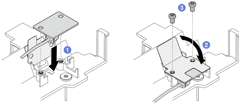
圖例 90. 安裝氣流感應器板
