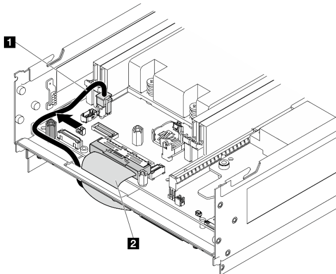
圖例 157. I/O 板纜線佈線
