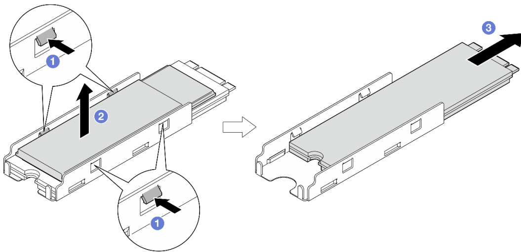
圖例 173. 卸下 M.2 散熱槽
