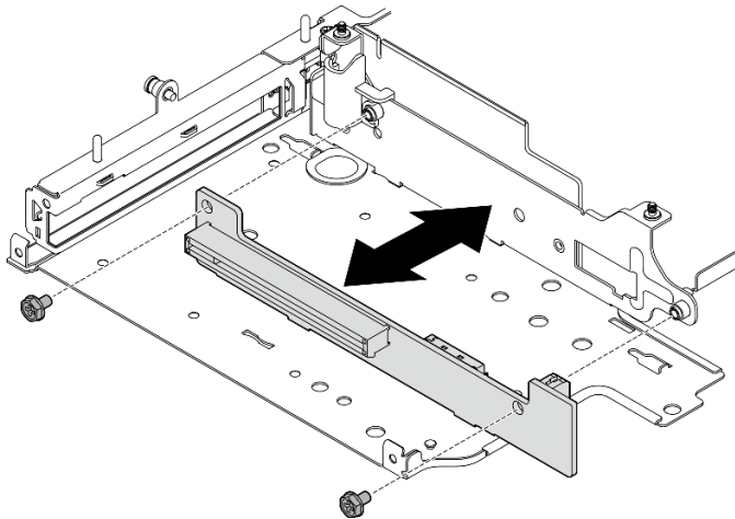
圖例 228. 卸下擴充卡
