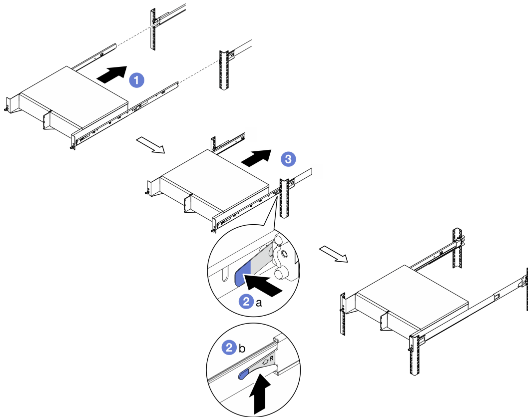
圖例 17. 將機體安裝到機架
