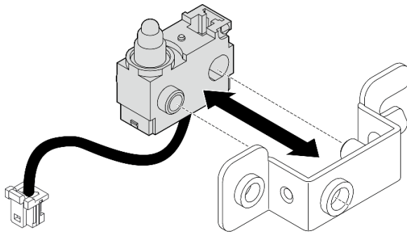
圖例 151. 將入侵開關插入托架
