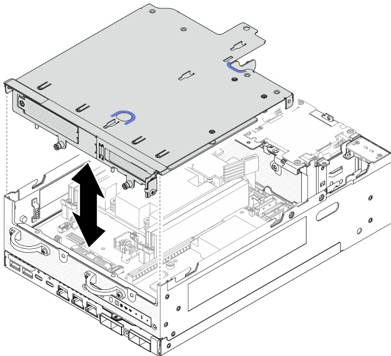
圖例 260. 放下擴充卡組件
