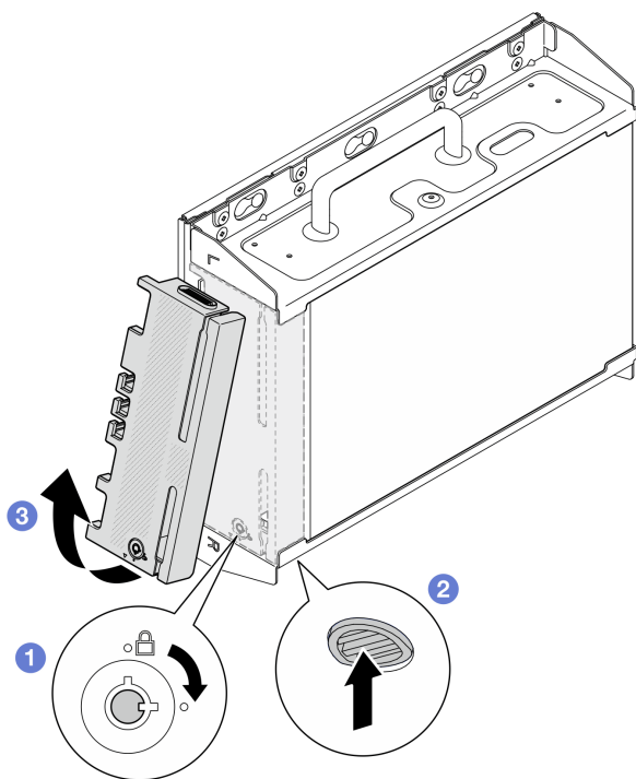
圖例 50. 卸下安全擋板
