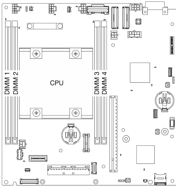
圖例 176. 記憶體模組和處理器佈置
