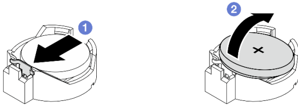
圖例 118. 取出 CMOS 電池
