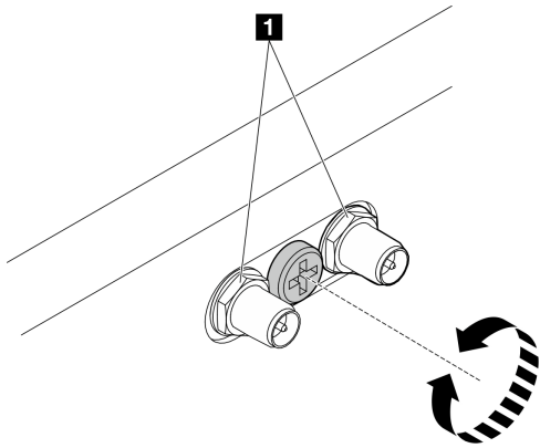
圖例 58. 縮短 SMA 接頭
