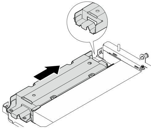
圖例 257. 安裝地理位置追蹤模組盒
