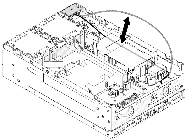
圖例 141. 放置信號線
