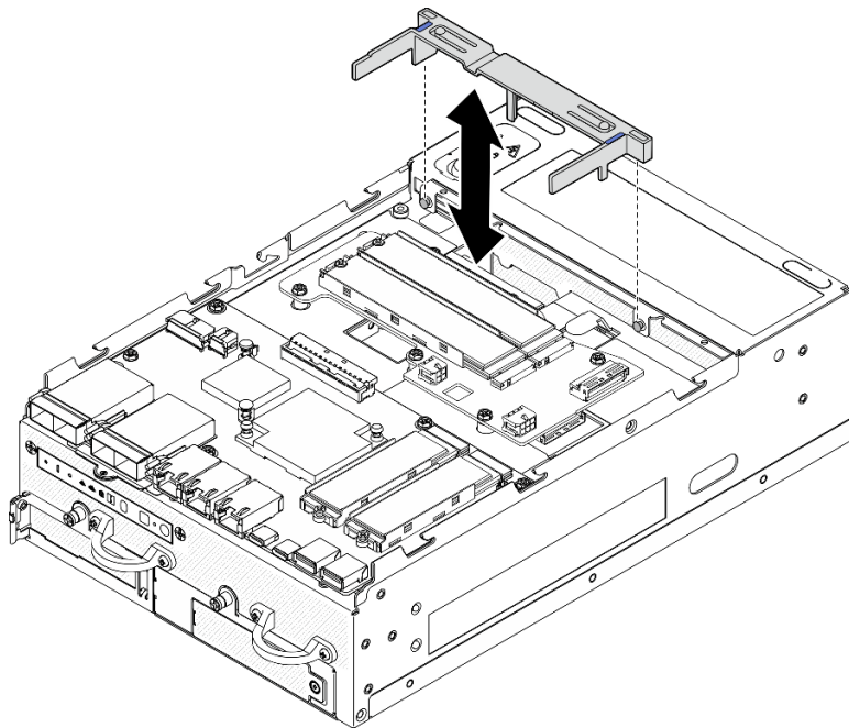
圖例 83. 安裝空氣擋板
