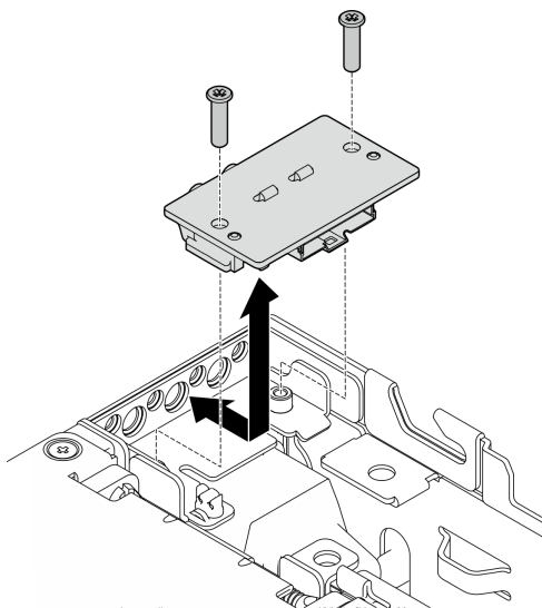
圖例 220. 卸下後方操作面板
