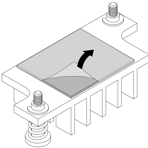
圖例 288. 取下散熱墊上的薄膜
