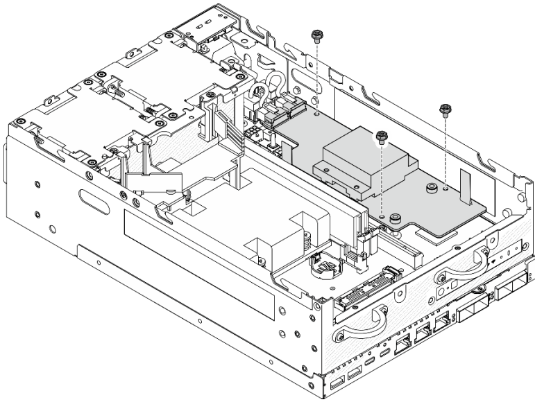
圖例 214. 固定電源模組板
