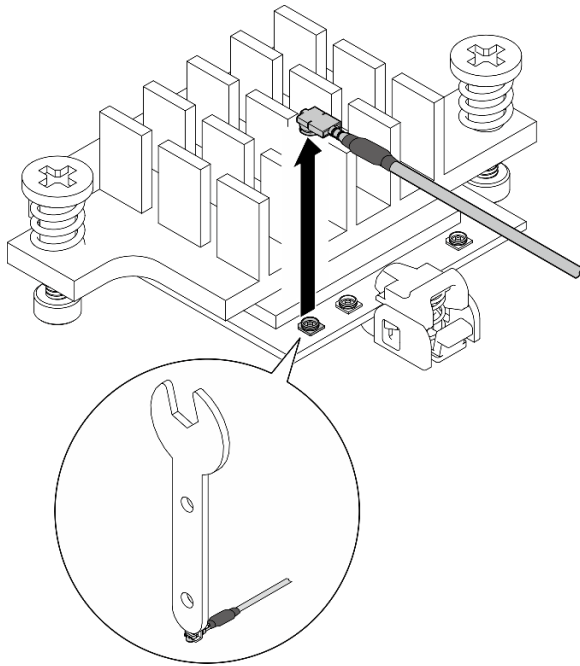
圖例 280. 拔下纜線
