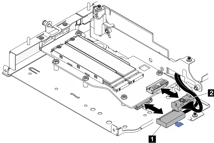
圖例 224. 拔掉信號線
