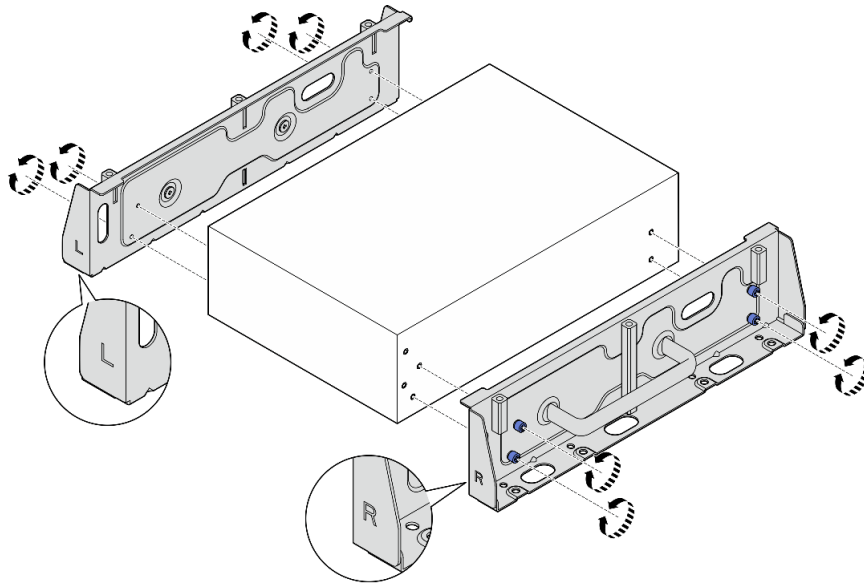
圖例 33. 鬆開翼型螺絲以卸下側托架
