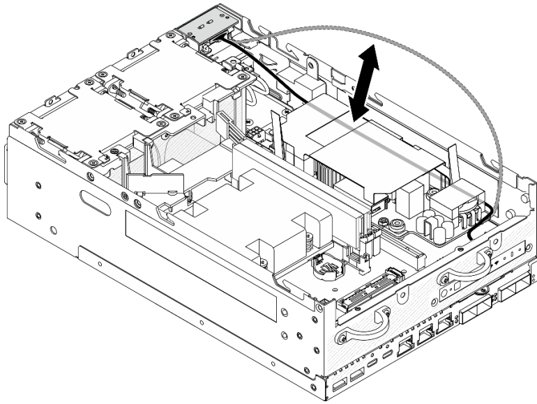
圖例 137. 放置信號線
