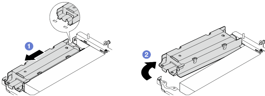
圖例 233. 卸下地理位置追蹤模組盒
