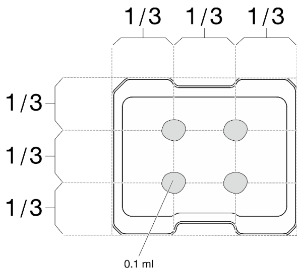
圖例 218. 散熱膏的適當形狀
