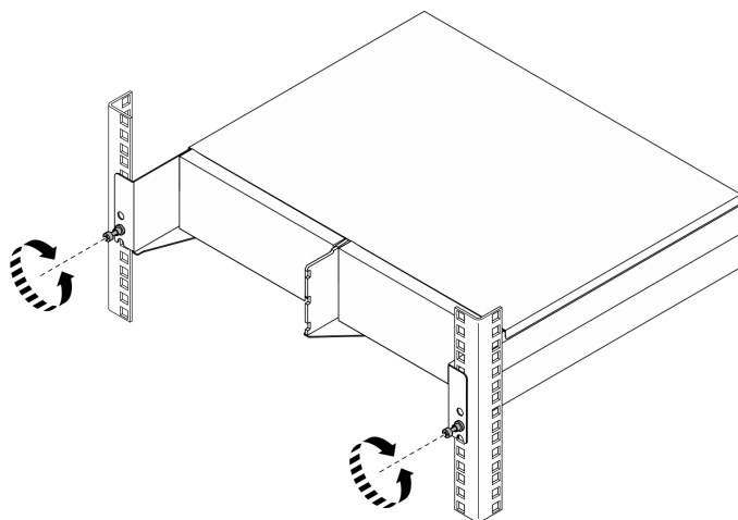
圖例 18. 將機體固定到機架
