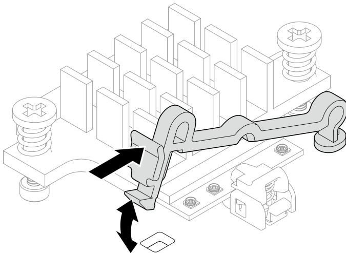
圖例 109. 插入纜線固定器
