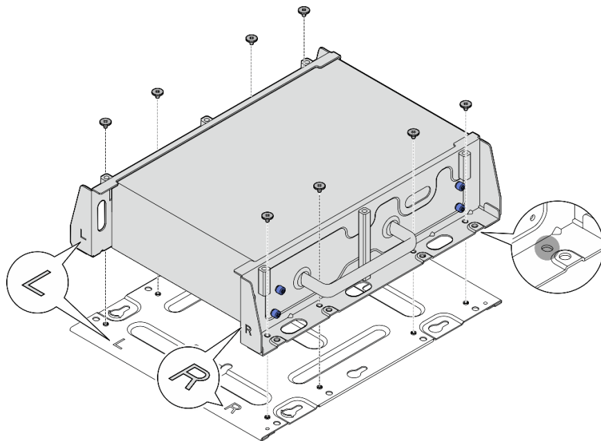
圖例 54. 卸下底板
