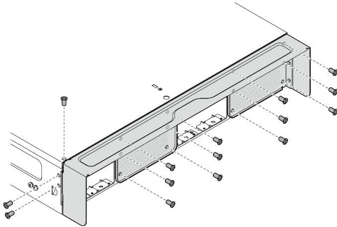
圖例 13. 鎖緊螺絲
