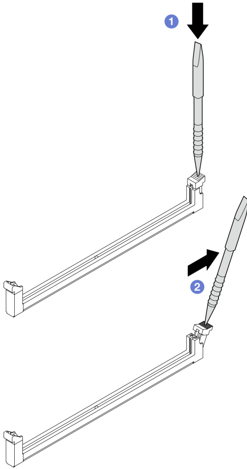
圖例 180. 打開固定夾
