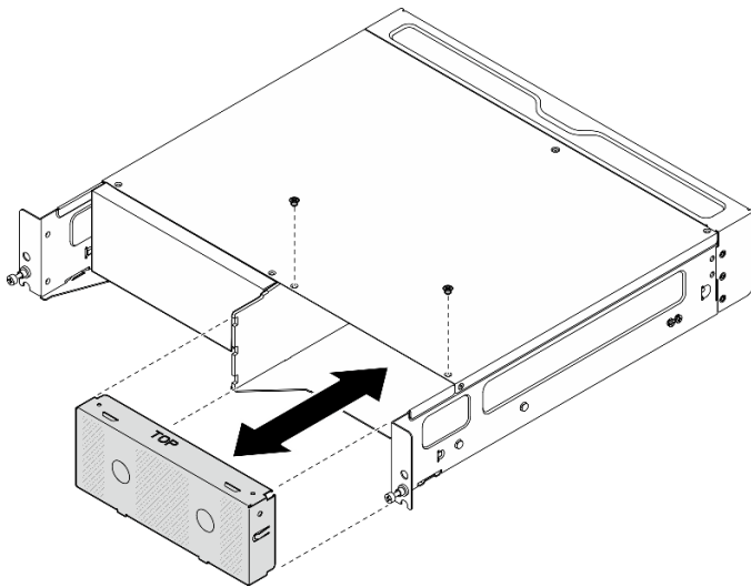
圖例 21. 卸下節點填充板
