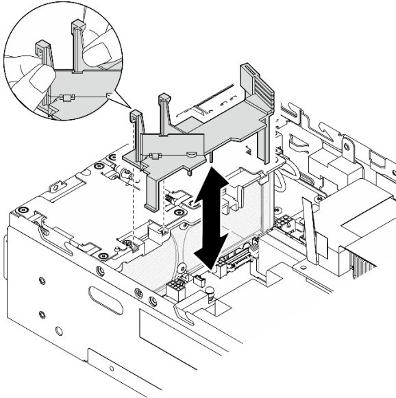
圖例 89. 安裝空氣擋板
