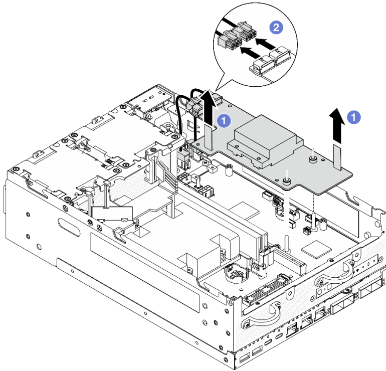
圖例 210. 卸下電源模組板
