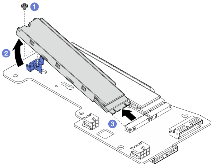
圖例 112. 卸下 M.2 硬碟
