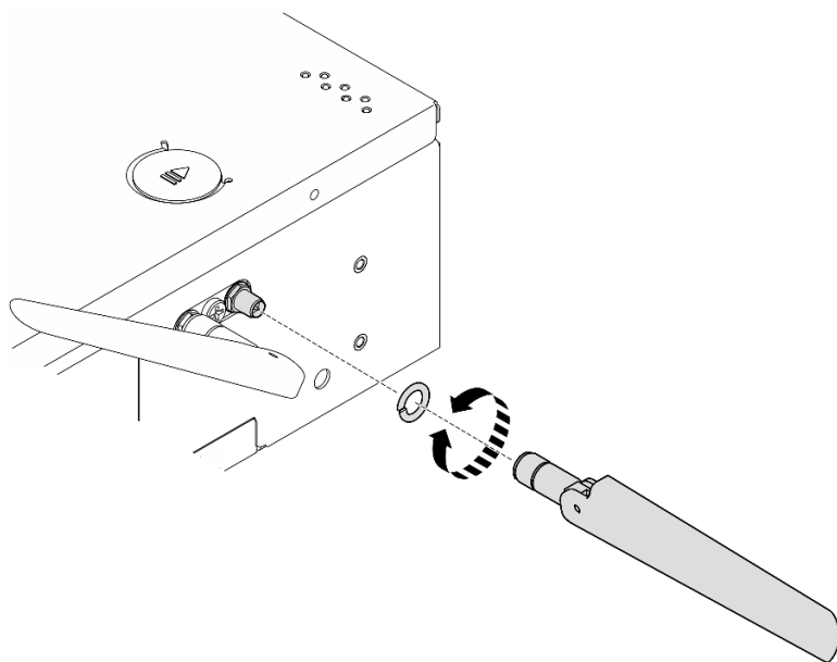
圖例 296. 卸下 WLAN 天線
