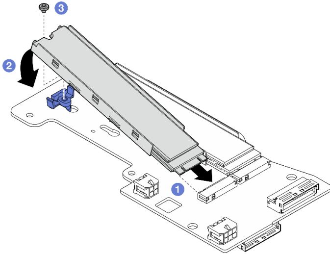
圖例 246. 安裝 M.2 硬碟
