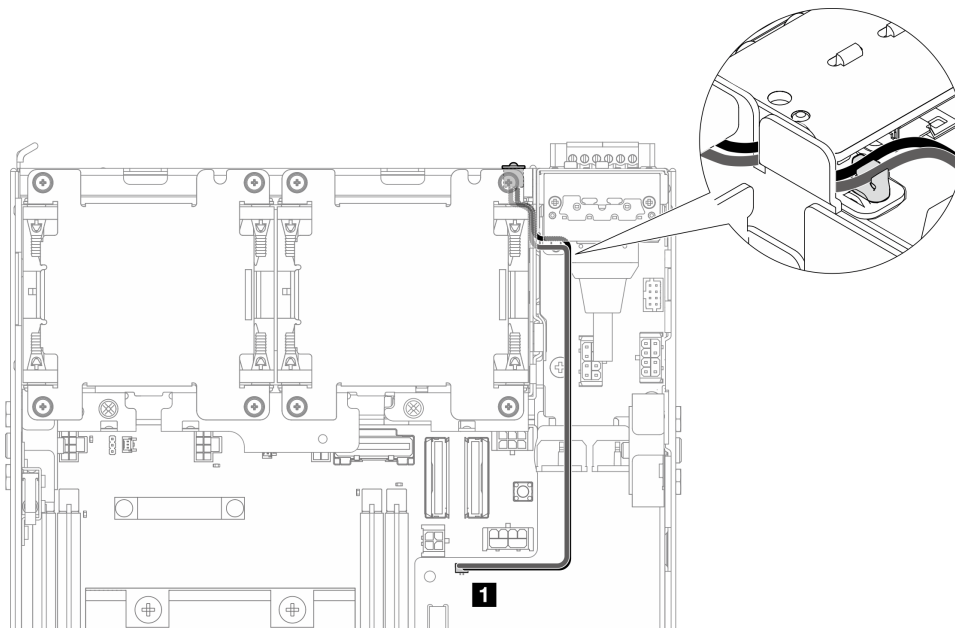
圖例 200. 連接到 DC 電源模組板 (DC PMB) 的 PMB 狀態 LED 纜線
