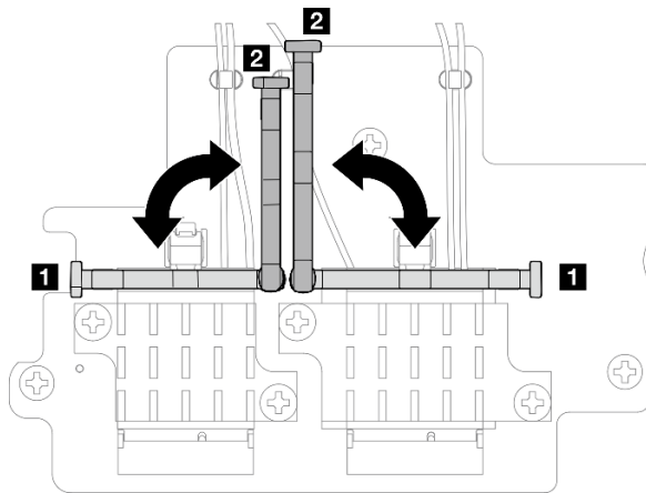
圖例 302. 轉動纜線固定器
