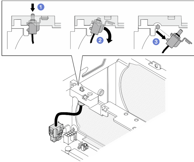
圖例 123. 卸下風扇方向開關
