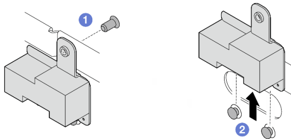
圖例 300. 卸下 SMA 填充板
