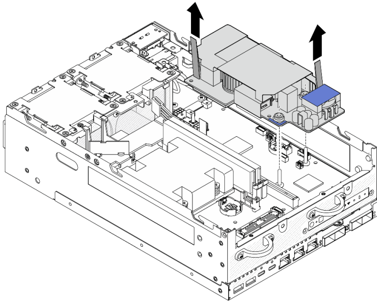
圖例 136. 卸下內部電源供應器
