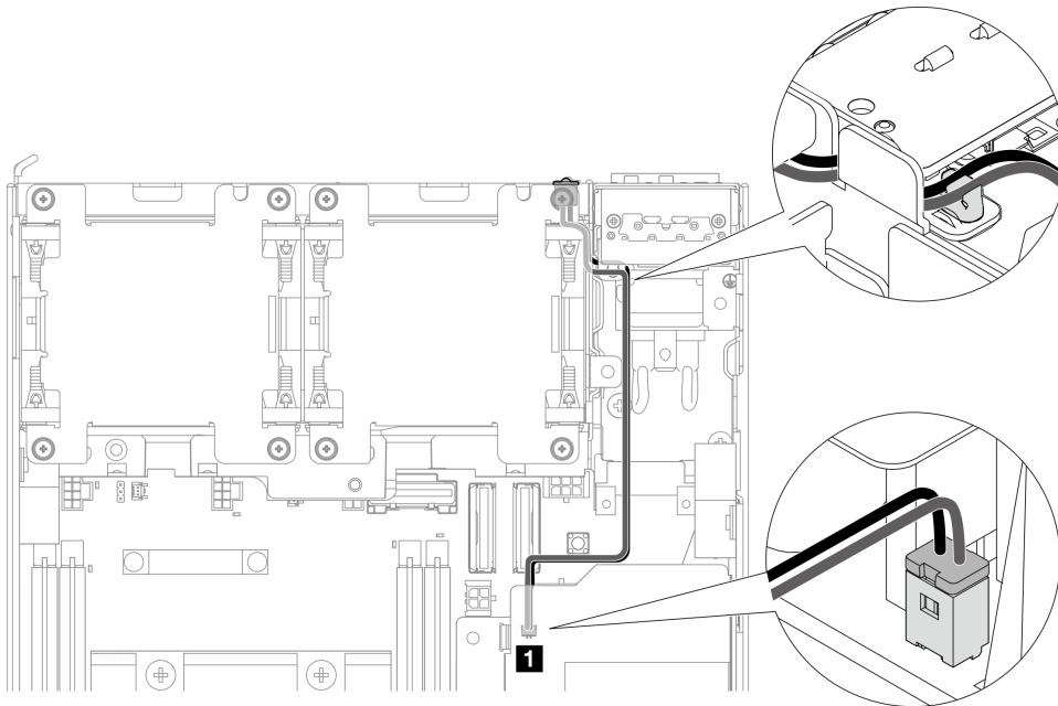
圖例 197. 連接到內部電源供應器 (AC PMB) 的 PMB 狀態 LED 纜線
