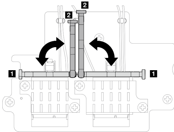
圖例 292. 轉動纜線固定器
