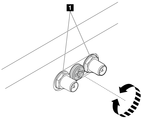
圖例 337. 伸出 SMA 接頭
