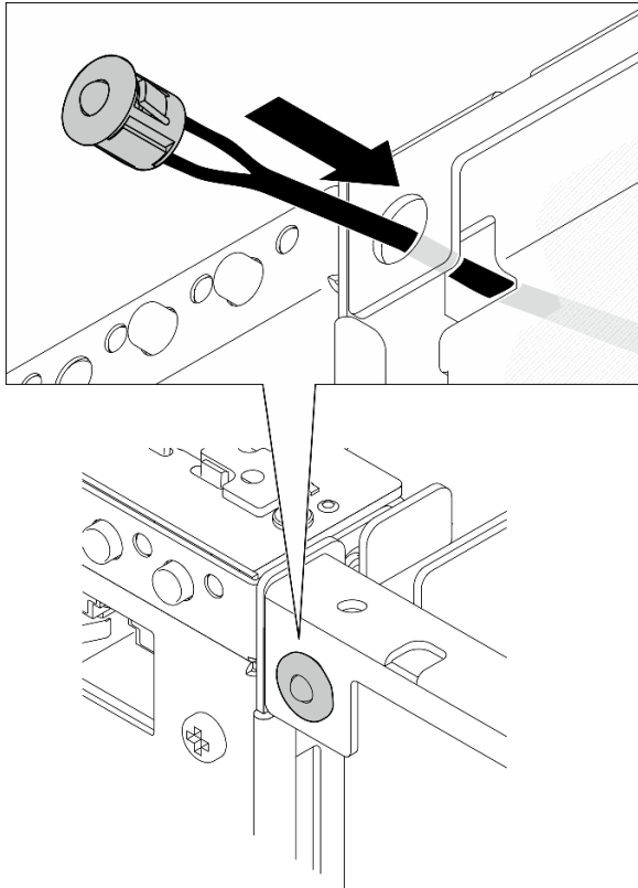
圖例 199. 安裝 PMB 狀態 LED 纜線
