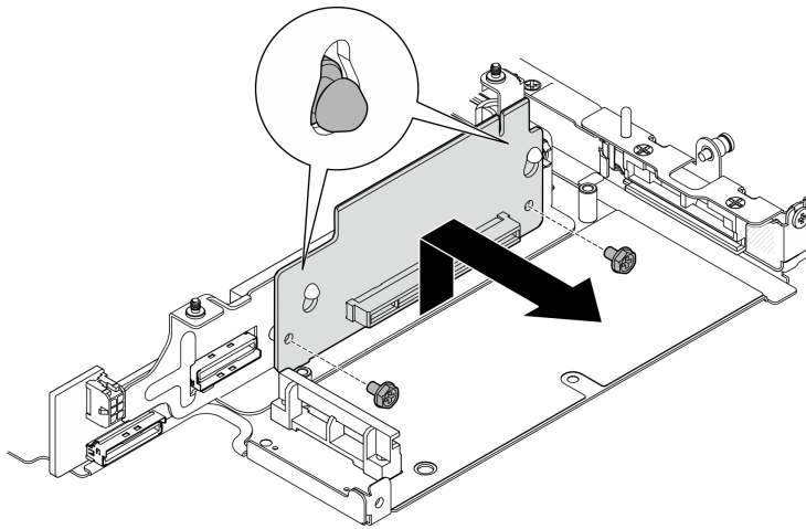
圖例 237. 卸下擴充卡
