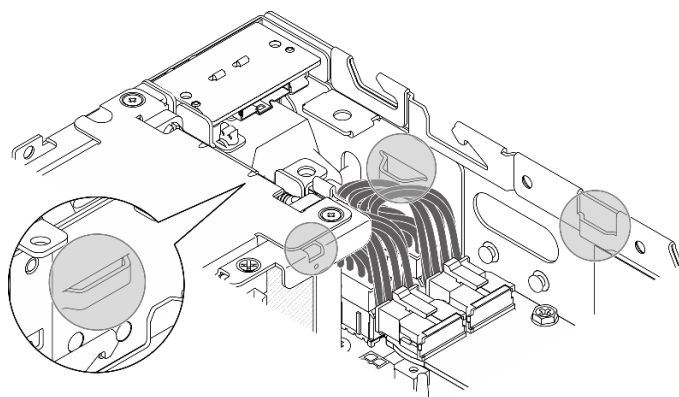
圖例 213. PMB 空氣擋板的插槽
