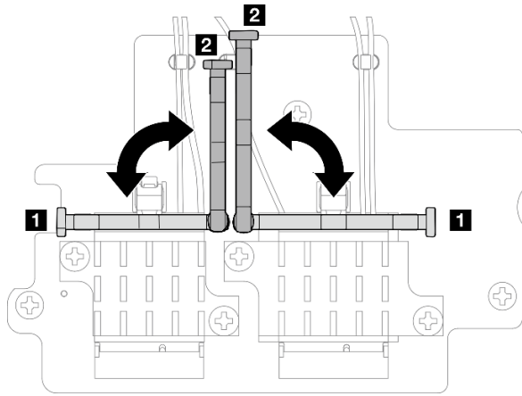
圖例 106. 轉動纜線固定器
