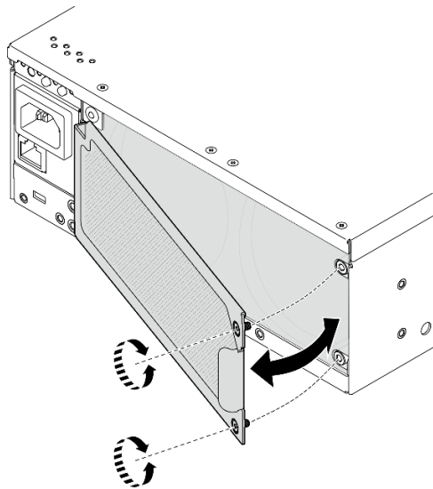
圖例 75. 安裝擋板
