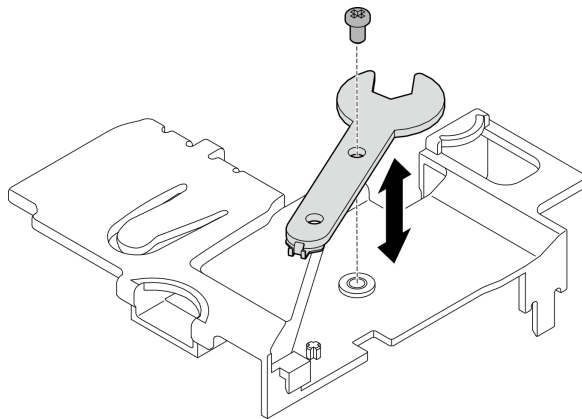
圖例 322. 鬆開扳手
