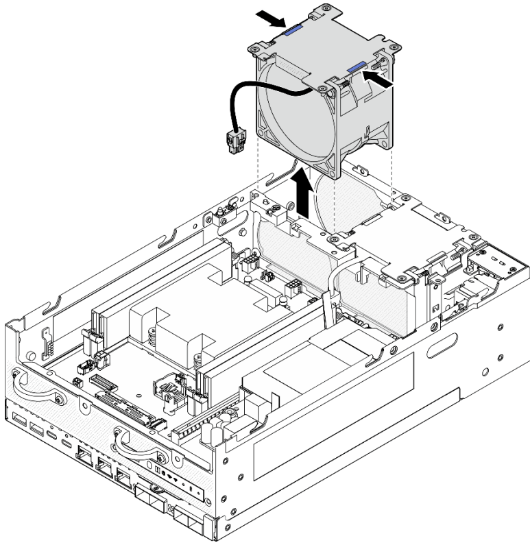
圖例 127. 卸下風扇模組
