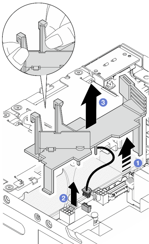
圖例 87. 卸下空氣擋板
