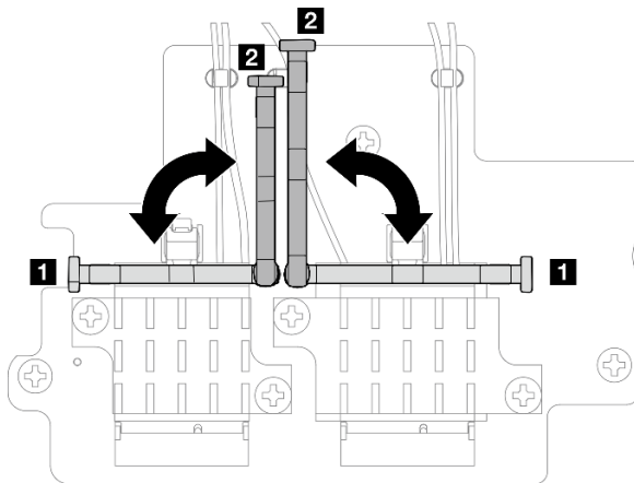
圖例 304. 轉動纜線固定器
