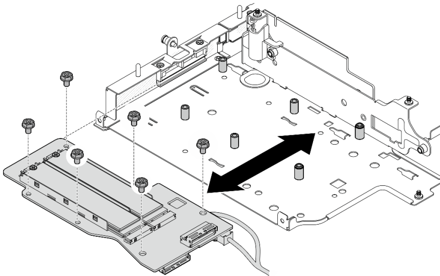
圖例 248. 安裝 M.2 配接卡
