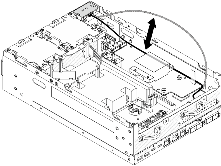
圖例 211. 放置信號線
