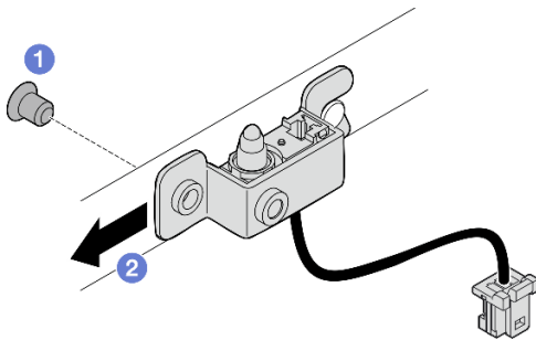
圖例 143. 卸下入侵開關及纜線
