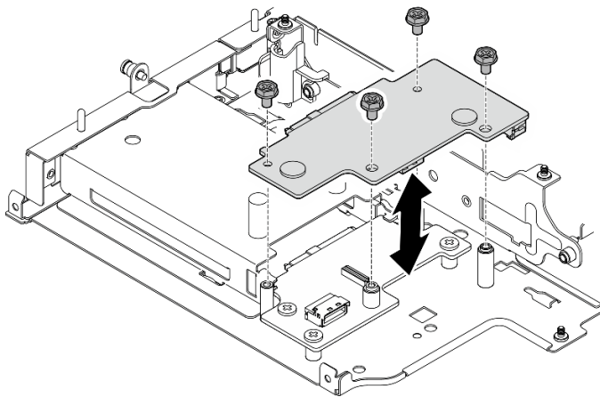
圖例 253. 安裝背板 2
