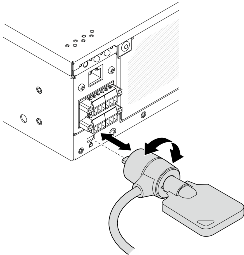
圖例 164. 安裝 Kensington 安全鎖
