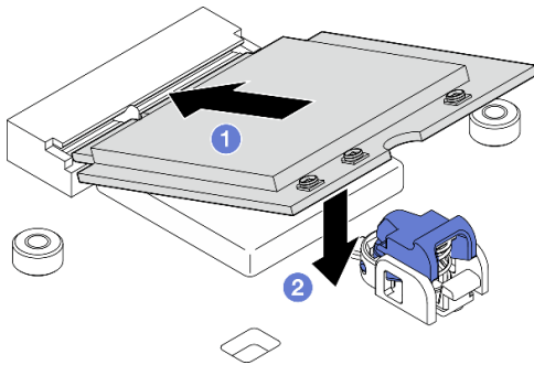
圖例 287. 安裝 WLAN/藍牙模組
