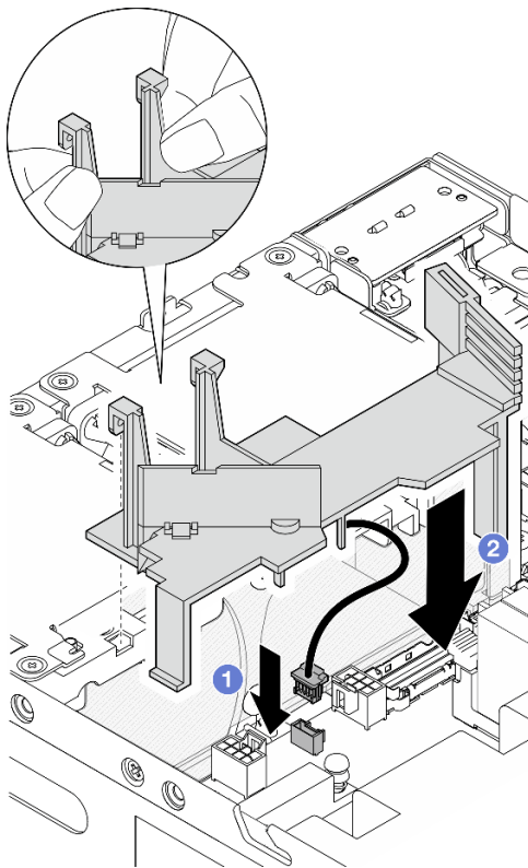
圖例 91. 安裝空氣擋板
