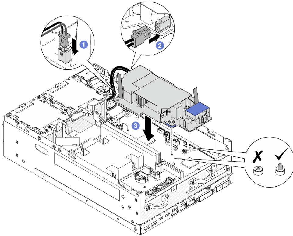
圖例 138. 安裝內部電源供應器
