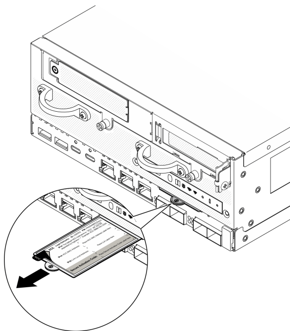
圖例 277. 拉出式資訊標籤上的 Lenovo XClarity Controller 網路存取標籤
