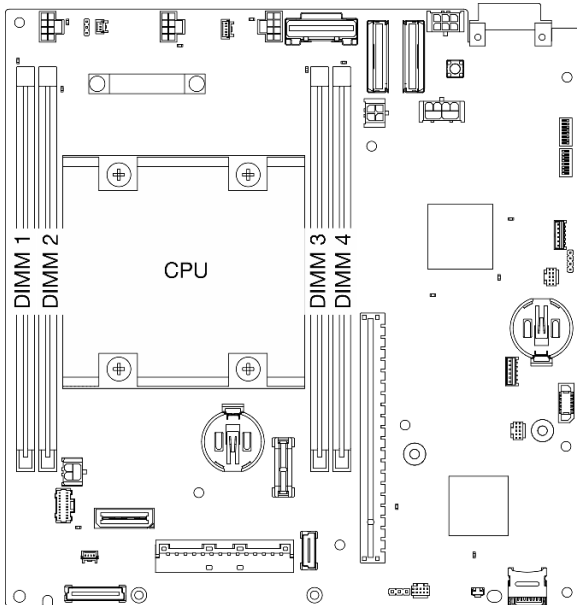
圖例 179. 記憶體模組和處理器佈置
