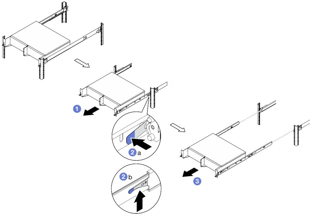
圖例 8. 從機架卸下機體
