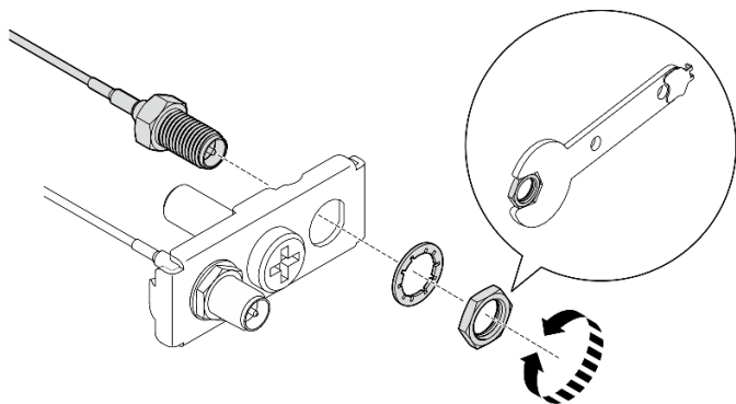
圖例 325. 將電纜固定在托架上
