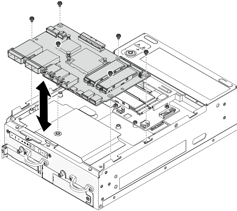
圖例 160. 安裝 I/O 模組板
