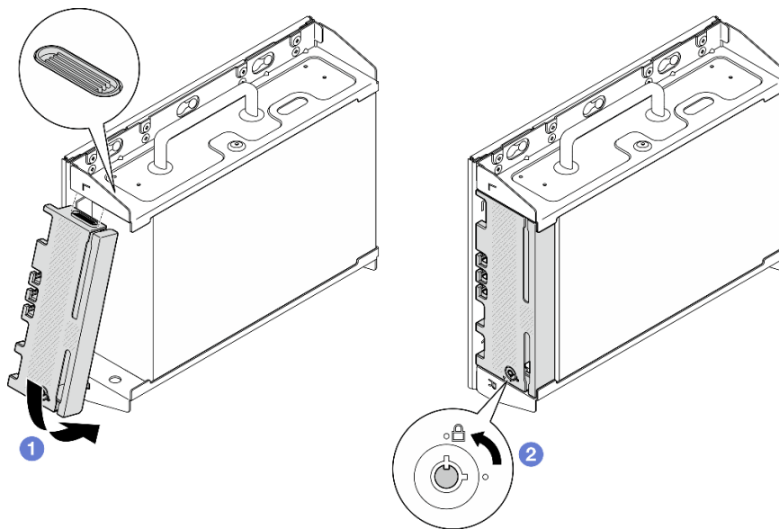
圖例 49. 安裝安全擋板
