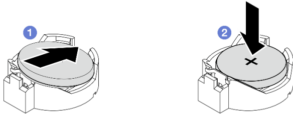
圖例 121. 安裝 CMOS 電池
