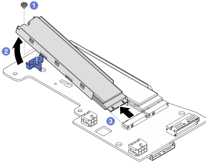
圖例 226. 卸下 M.2 硬碟
