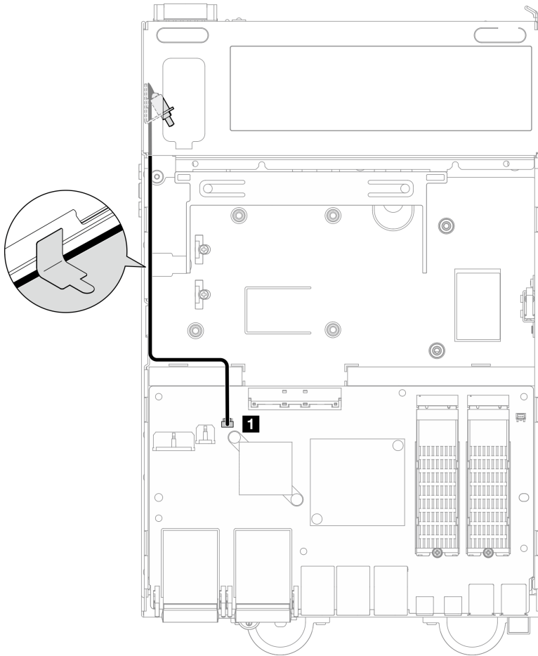
圖例 167. 鎖定位置開關纜線佈線
