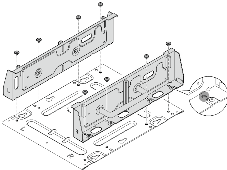
圖例 59. 拆卸節點托架
