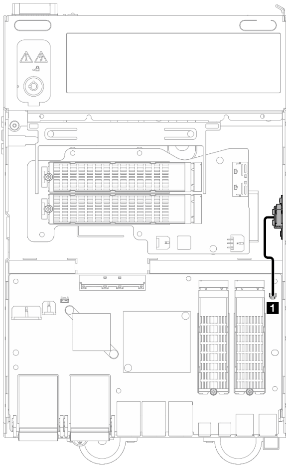
圖例 153. 底部入侵開關纜線佈線
