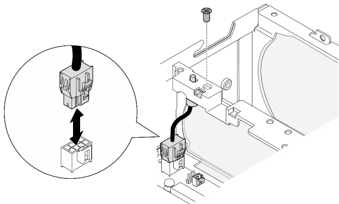
圖例 122. 卸下風扇方向開關
