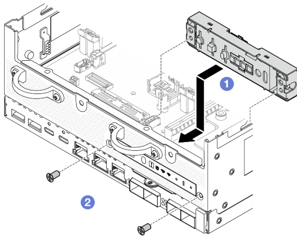
圖例 131. 安裝前方操作面板
