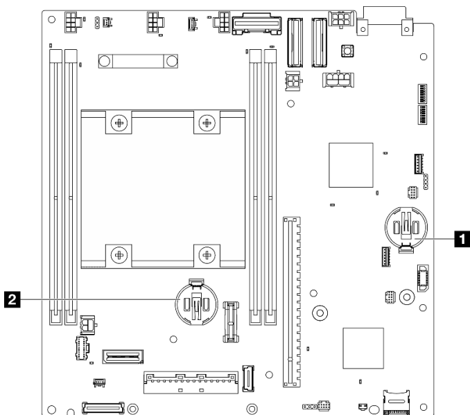
圖例 120. 主機板上的 CMOS 電池位置
