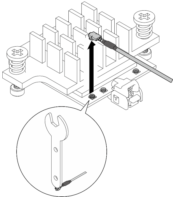
圖例 314. 拔下纜線
