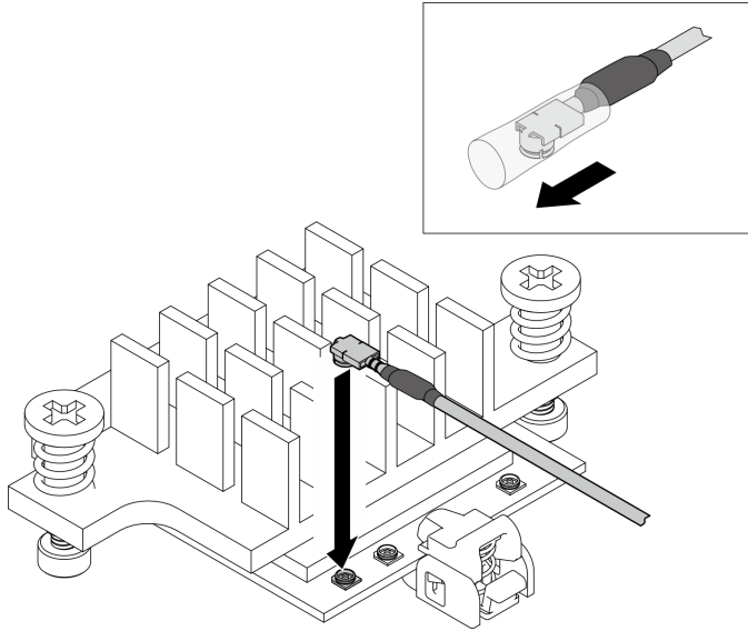
圖例 331. 連接纜線
