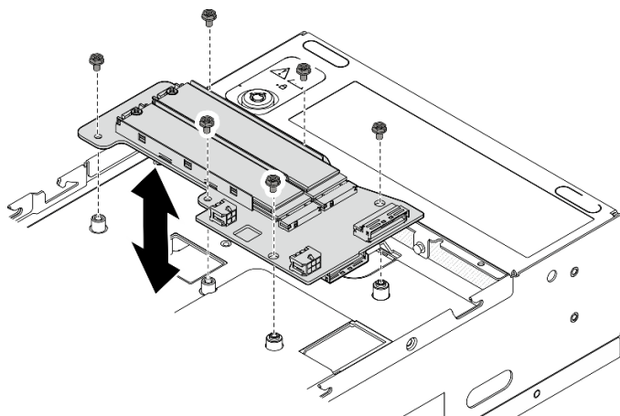
圖例 115. 安裝底部 M.2 含纜線配接卡
