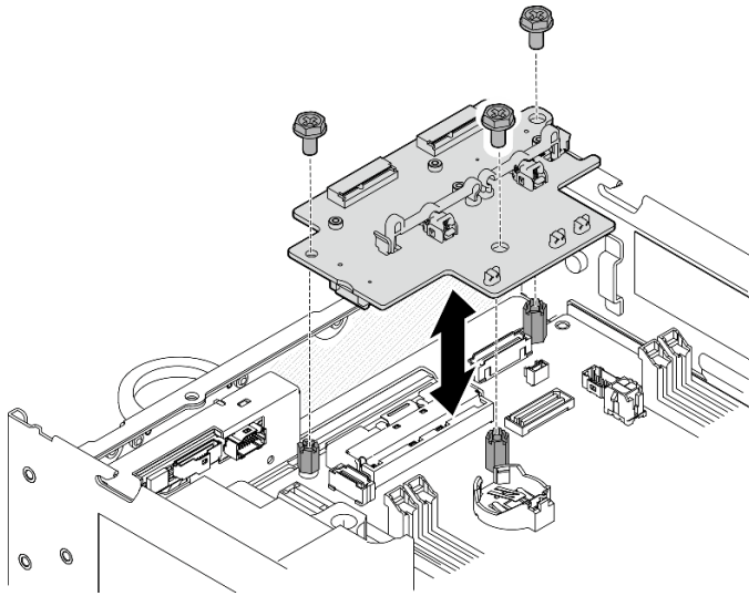
圖例 283. 卸下無線配接卡
