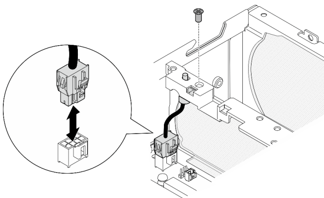
圖例 125. 安裝風扇方向開關
