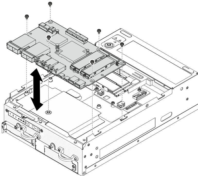
圖例 155. 卸下 I/O 模組板
