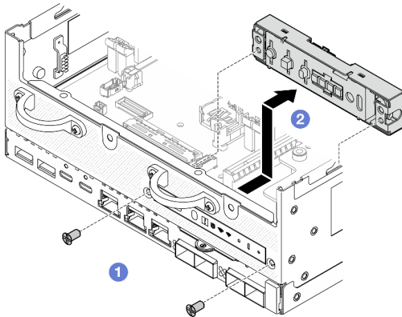
圖例 130. 卸下前方操作面板
