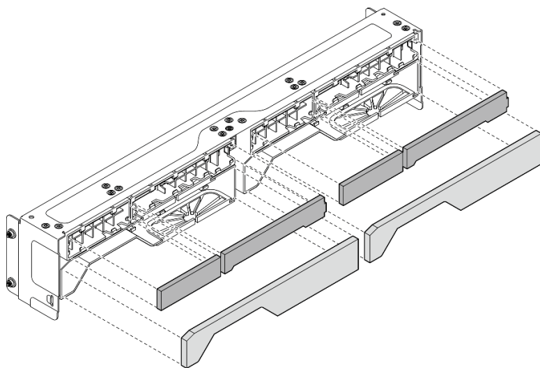
圖例 69. 安裝灰塵過濾器
