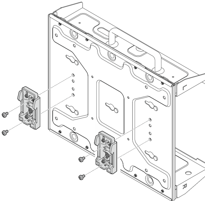
圖例 63. 安裝 DIN 滑軌固定夾
