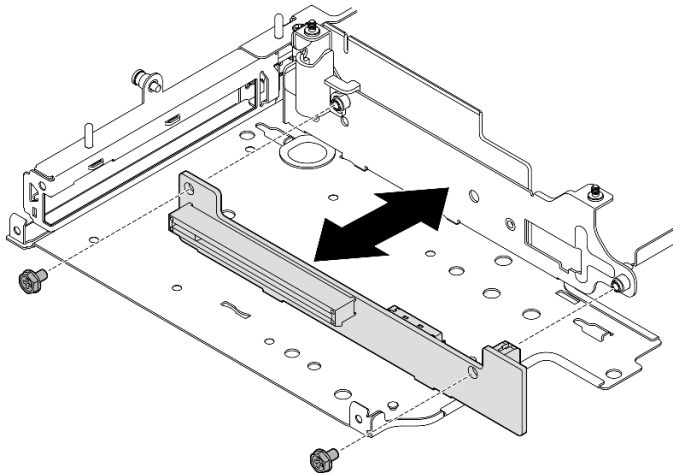
圖例 235. 卸下擴充卡
