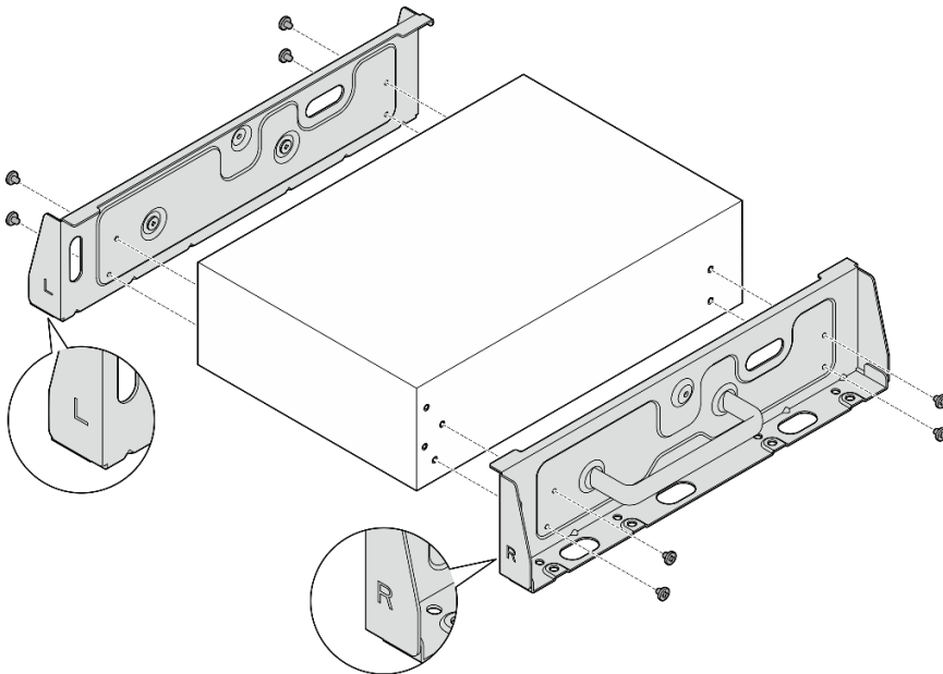
圖例 32. 鬆開螺絲以卸下側托架
