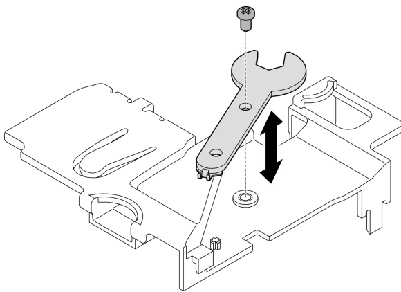
圖例 111. 存放扳手
