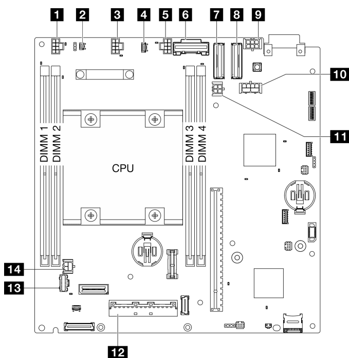
圖例 340. 主機板接頭
