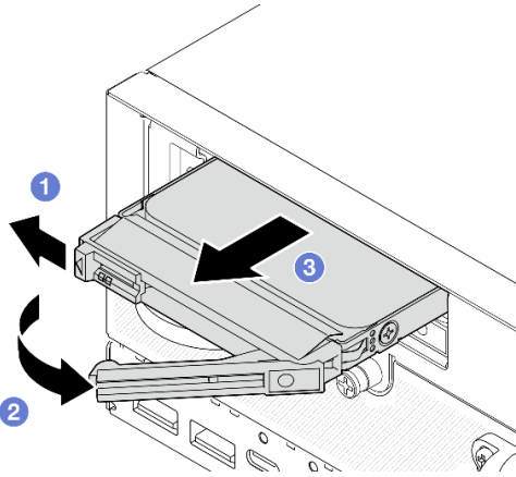
圖例 77. 卸下 7 公釐硬碟
