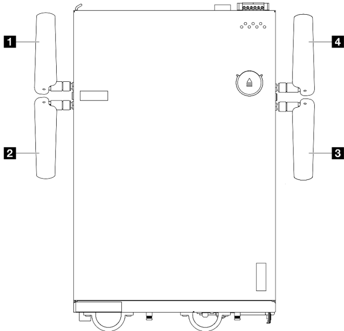
圖例 336. WLAN 天線的位置
