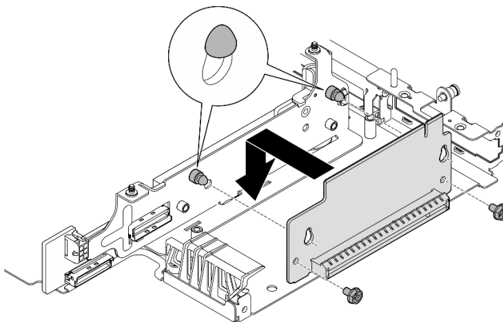
圖例 244. 安裝擴充卡
