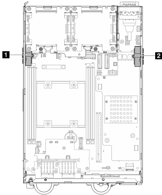
圖例 297. SMA 組件位置
