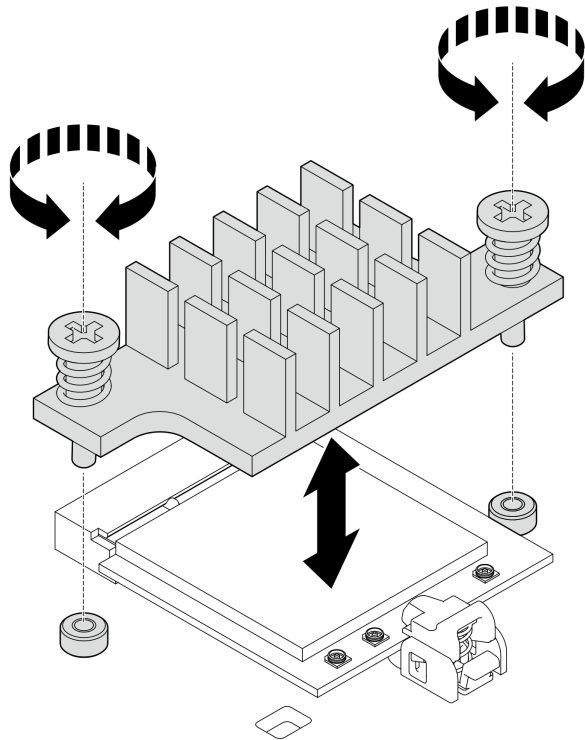
圖例 289. 安裝 WLAN/藍牙模組散熱槽
