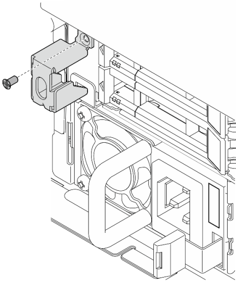
Abbildung 179. Halterung für Schlüsselhalterung für Sicherheitsfrontblende installieren
