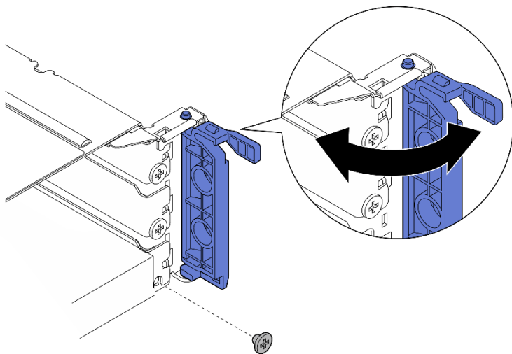
Abbildung 126. Unverlierbare Schrauben installieren
