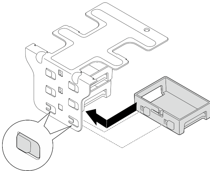
Abbildung 129. Flache Abdeckblende installieren
