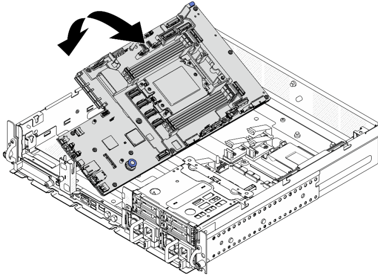
Abbildung 188. Installieren der Systemplatine
