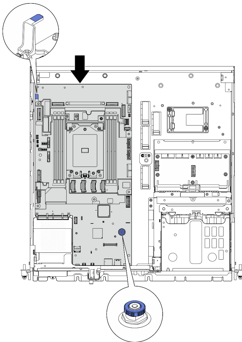
Abbildung 189. Sichern der Systemplatine
