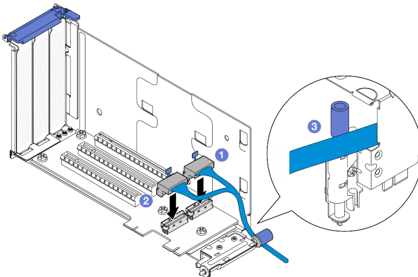
Abbildung 145. Kabelführung für PCIe-Adapterkarte 1
