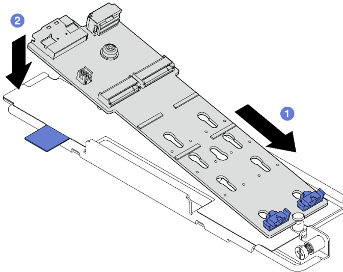
Abbildung 88. M.2-Rückwandplatine installieren
