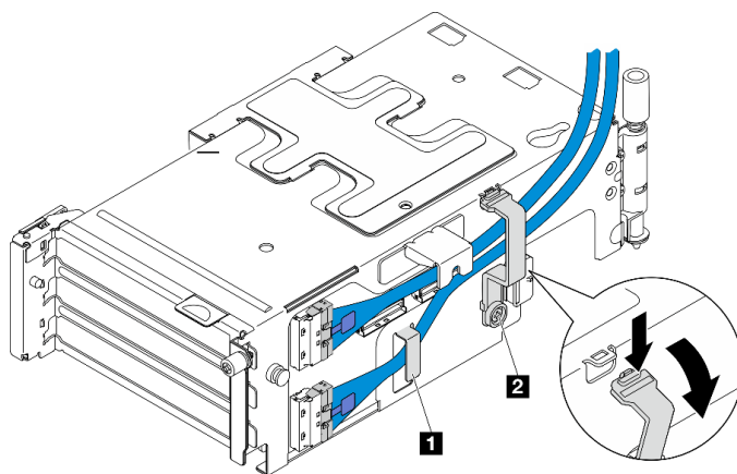
Abbildung 148. Kabelführung für PCIe-Adapterkarte 2
