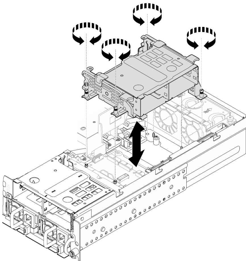
Abbildung 70. Interne Laufwerkhalterung installieren
