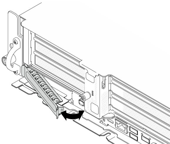
Abbildung 104. Entfernen der OCP-Abdeckblende
