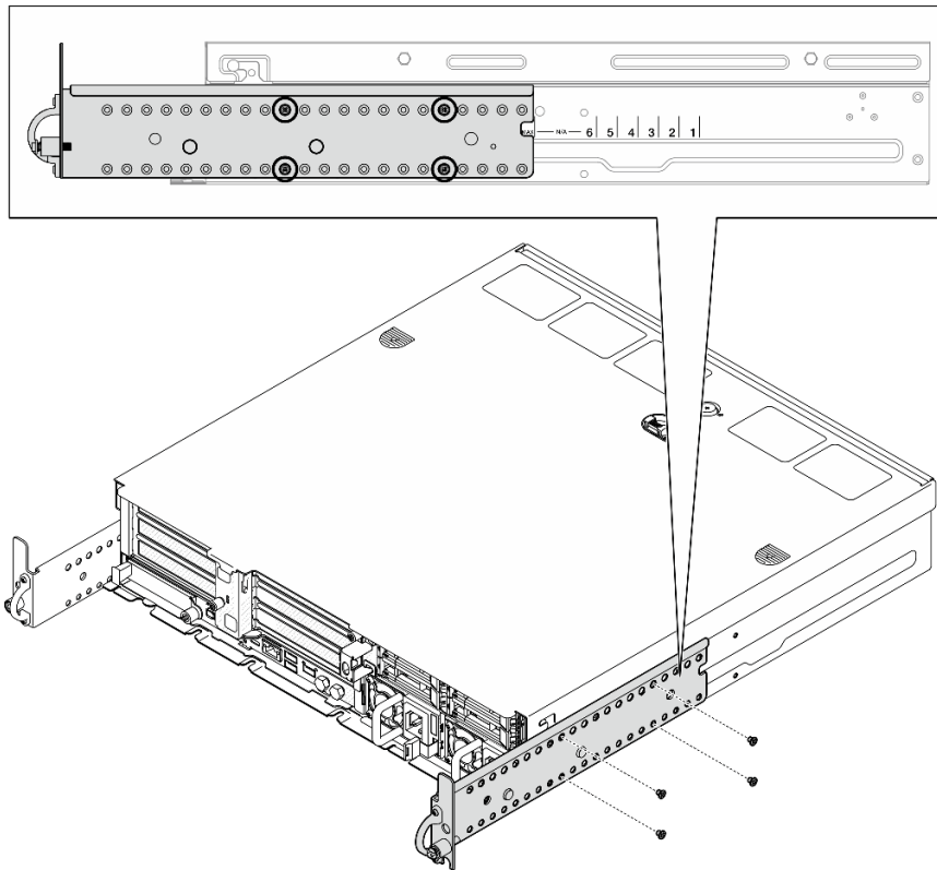
Abbildung 15. EIA-Halterung mit maximaler Tiefe für Sicherheitsfrontblende: vier Schrauben
