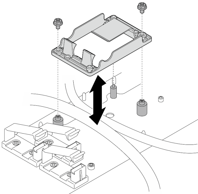
Abbildung 168. Halterung des RAID-Flash-Stromversorgungsmoduls entfernen
