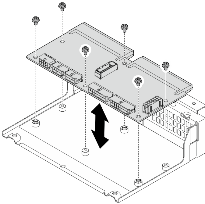
Abbildung 153. Installieren der Stromversorgungsplatine
