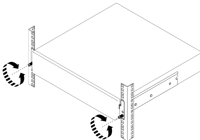
Abbildung 23. Sichern des Servers an der Vorderseite des Racks: Standard-EIA-Halterungen
