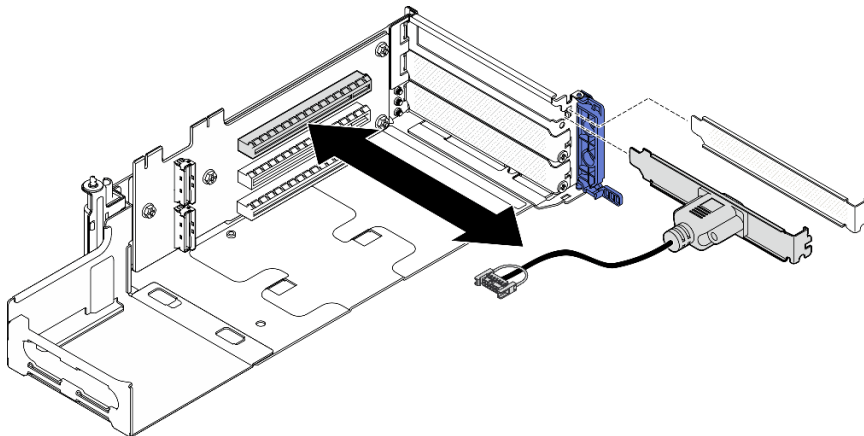
Abbildung 182. Serielles Anschlussmodul installieren
