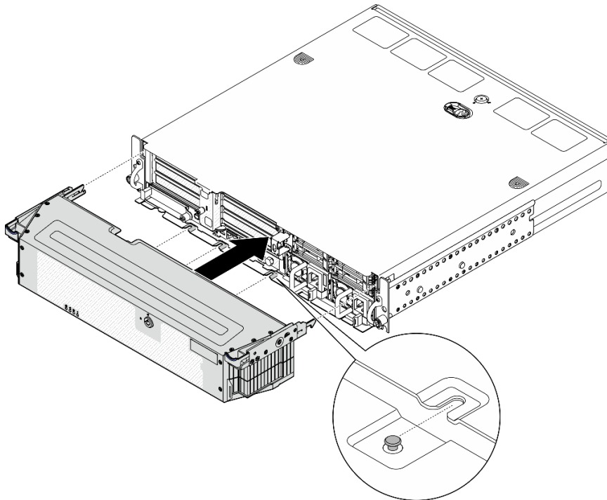
Abbildung 175. Installieren der Sicherheitsfrontblende
