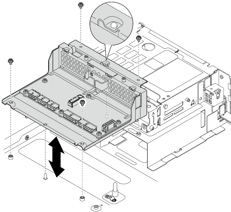
Abbildung 151. PDB-Gehäuse entfernen
