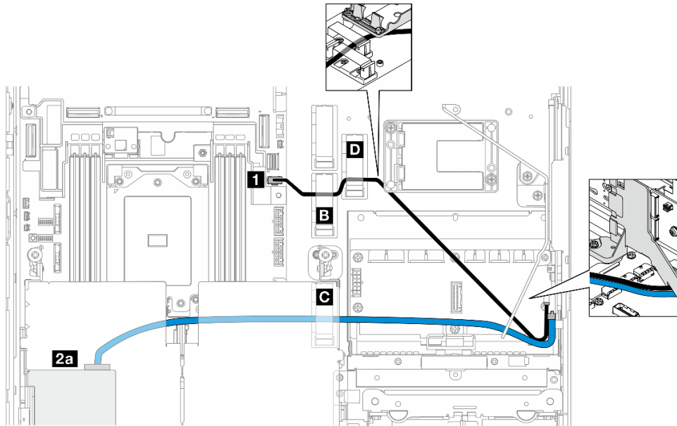
Abbildung 206. RAID-Adapter auf PCIe-Adapterkarte 1
