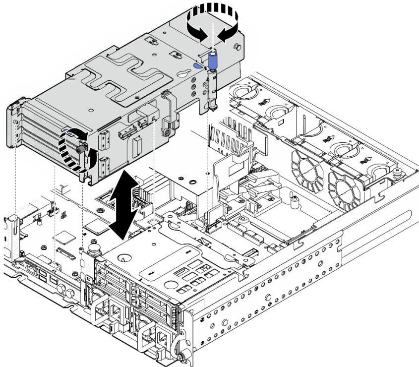
Abbildung 113. PCIe-Adapterkarte 2 hochheben
