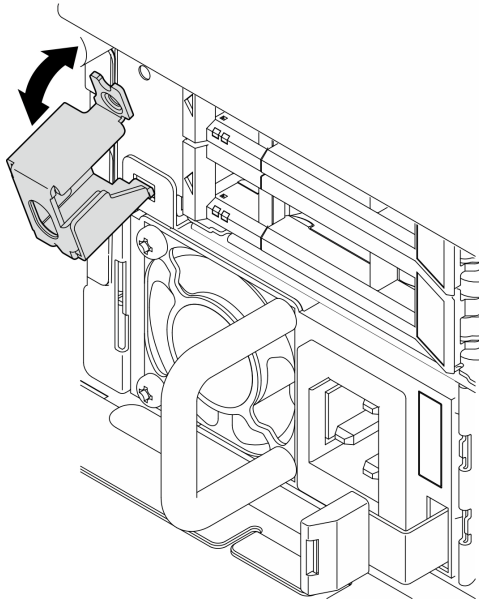
Abbildung 177. Schlüsselhalterung für Sicherheitsfrontblende entfernen
