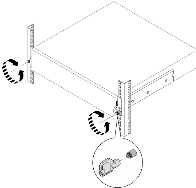
Abbildung 24. Sichern des Servers an der Vorderseite des Racks: Sicherheits-EIA-Halterungen
