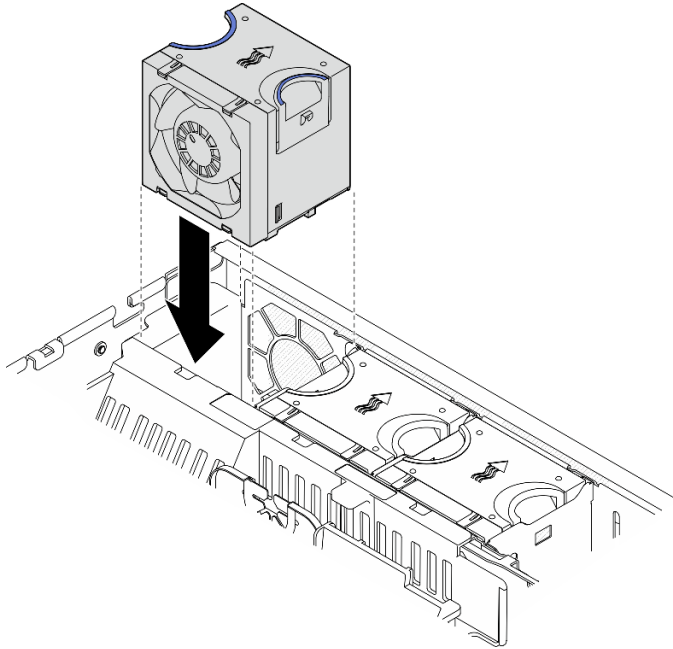
Abbildung 49. Installieren eines Lüfters
