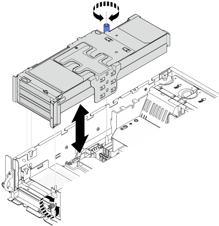
Abbildung 132. Installieren von PCIe-Adapterkarte 1
