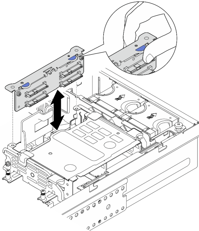
Abbildung 66. Interne Rückwandplatine entfernen
