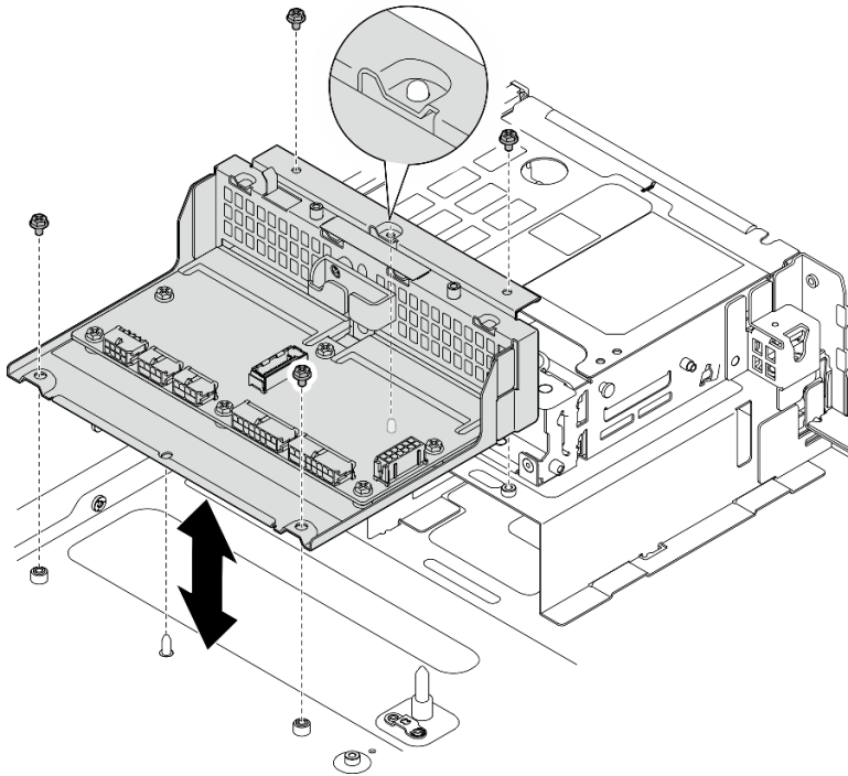
Abbildung 152. PDB-Gehäuse installieren
