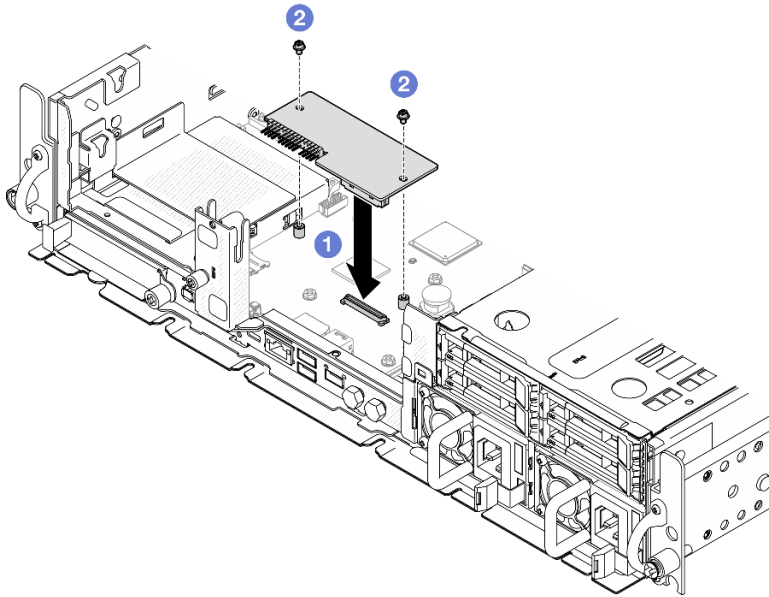
Abbildung 185. Installieren des Firmware- und RoT-Sicherheitsmoduls
