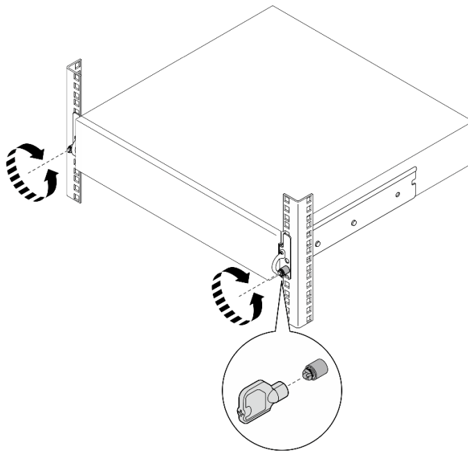
Abbildung 3. Trennen des Servers aus dem Rack: Sicherheits-EIA-Halterungen
