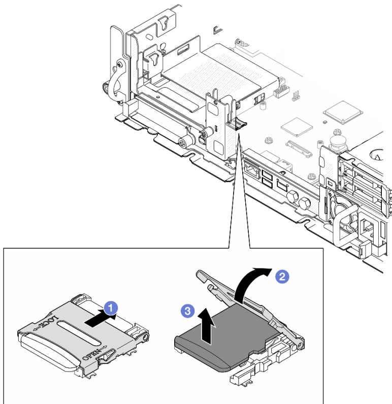
Abbildung 100. Entfernen der microSD-Karte
