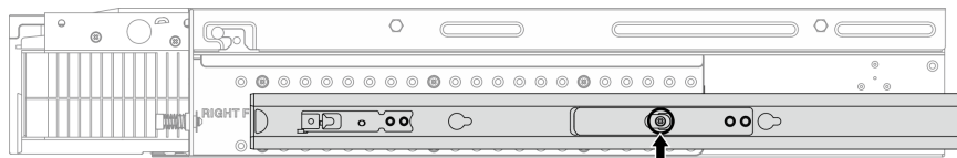
Abbildung 8. Eine Schraube für die innere Schiene der ThinkEdge 2-Pfosten-Reibungsschienenatz
