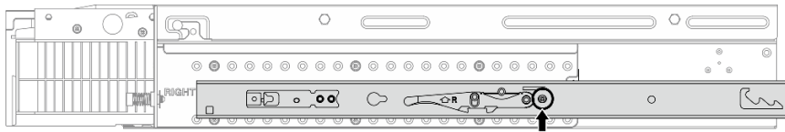
Abbildung 18. Eine Schraube für die innere Schiene des ThinkEdge Kugellager-Schienensatz für 600-mm-Rack
