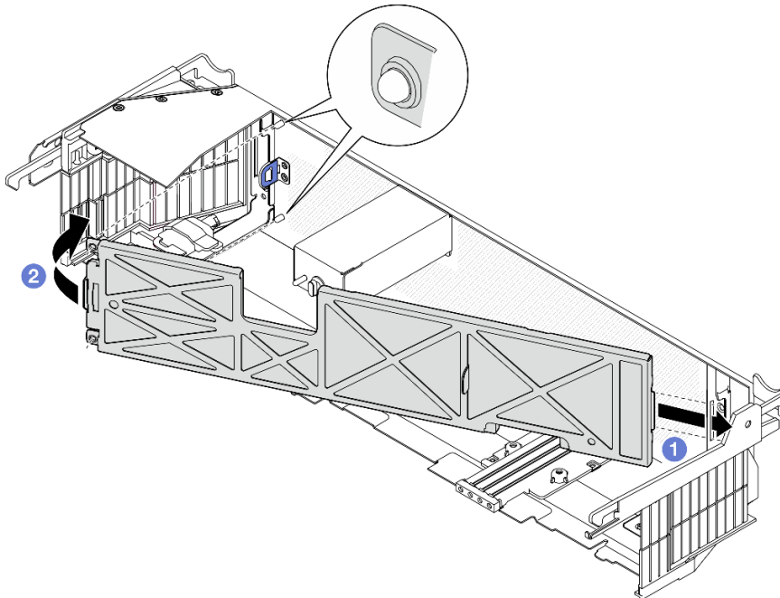
Abbildung 173. Installieren des Staubfilters
