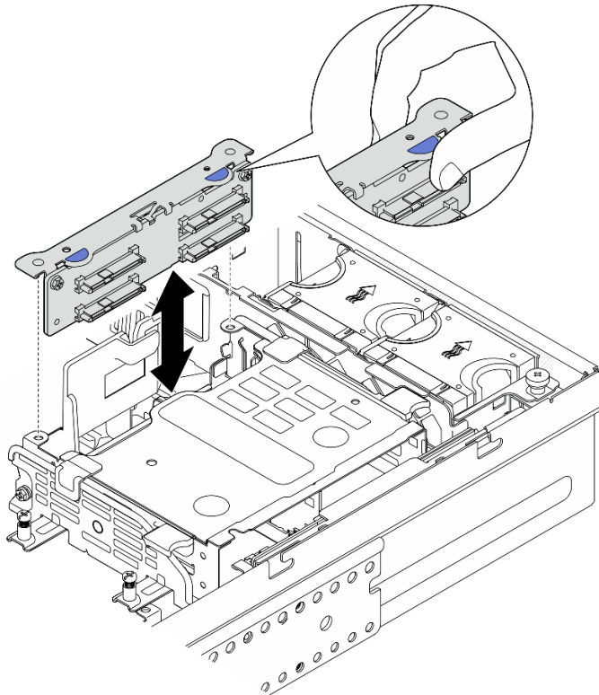
Abbildung 111. Interne Rückwandplatine entfernen
