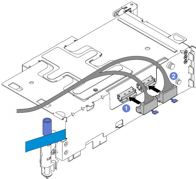
Abbildung 146. Kabelführung für PCIe-Adapterkarte 1
