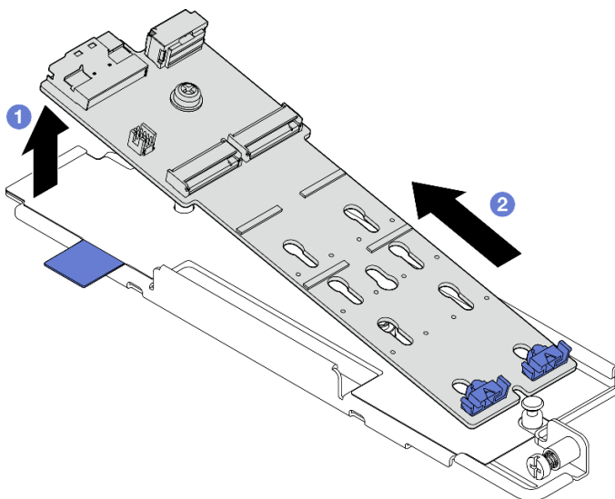
Abbildung 87. M.2-Rückwandplatine entfernen
