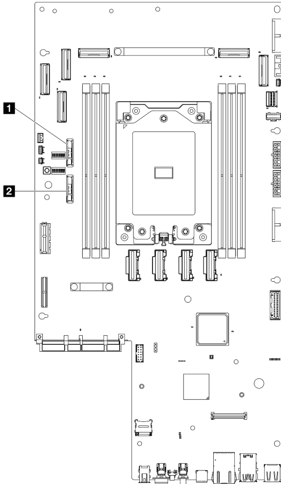
Abbildung 46. Positionen der CMOS-Batterie auf der Systemplatine
