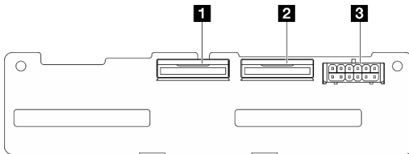
Abbildung 195. NVMe-Rückwandplatine
