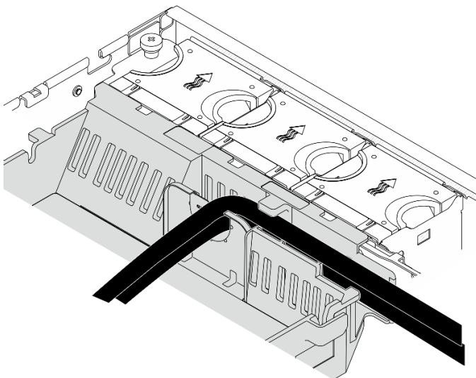
Abbildung 112. GPU-Netzkabel an der Prozessorluftführung
