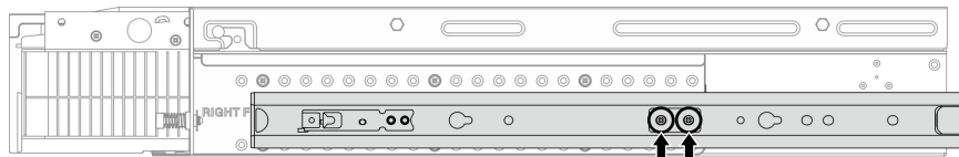
Abbildung 9. Zwei Schrauben für die innere Schiene der ThinkEdge 1.000 mm Schienenatz v2
