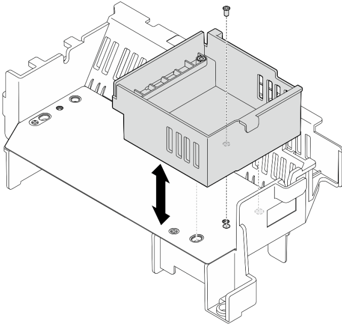
Abbildung 34. Abdeckblende für die Adapterkarte 2 austauschen
