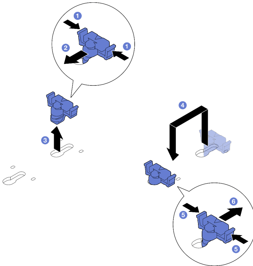
Abbildung 90. M.2-Halterung anpassen
