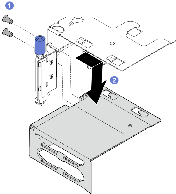
Abbildung 121. Extender aus PCIe-Adapterkarte 2 entfernen
