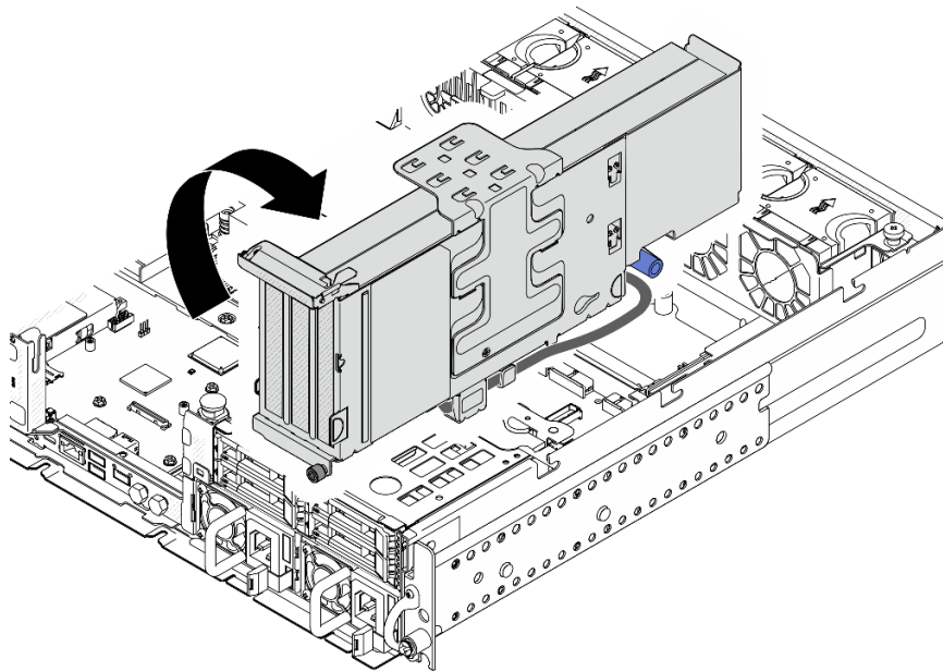
Abbildung 114. PCIe-Adapter 2 neben dem Gehäuse platzieren
