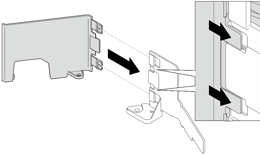
Abbildung 28. Teile der M.2-Luftführung kombinieren
