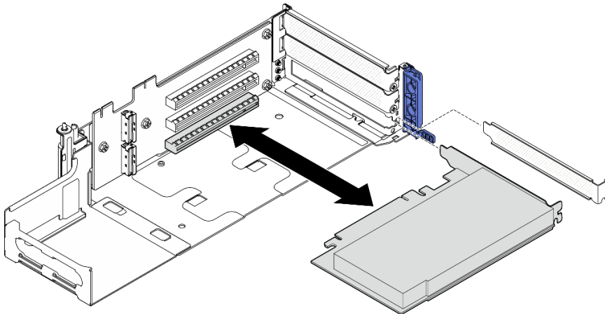
Abbildung 118. PCIe-Adapter aus PCIe-Adapterkarte 1 entfernen
