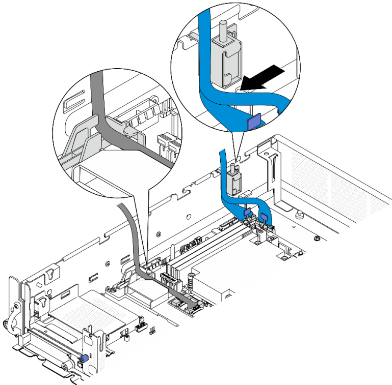
Abbildung 131. Kabelführung für PCIe-Adapterkarte 1
