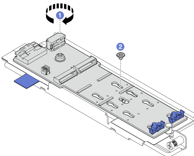
Abbildung 89. M.2-Rückwandplatine installieren
