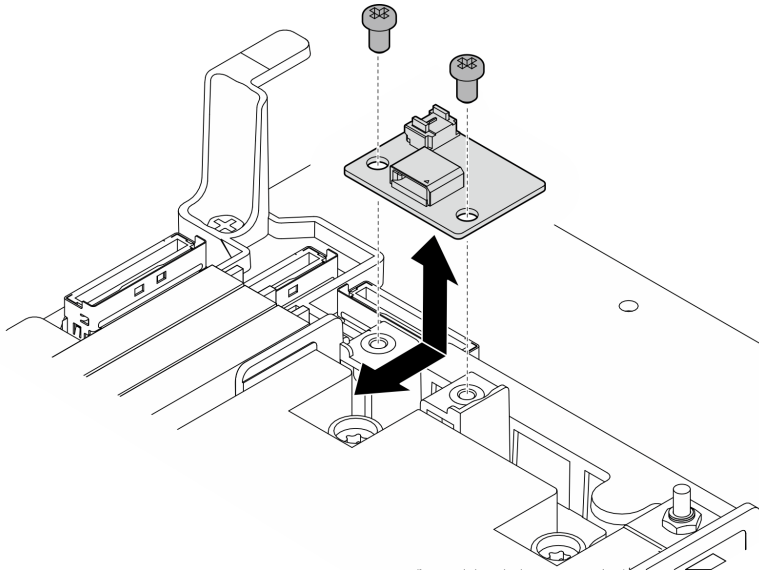
Abbildung 39. Installieren der Luftmassensensorplatine
