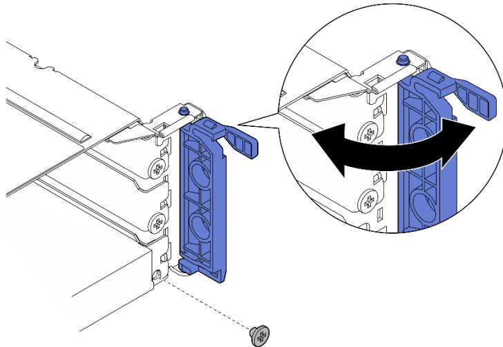
Abbildung 117. Halteschraube entfernen
