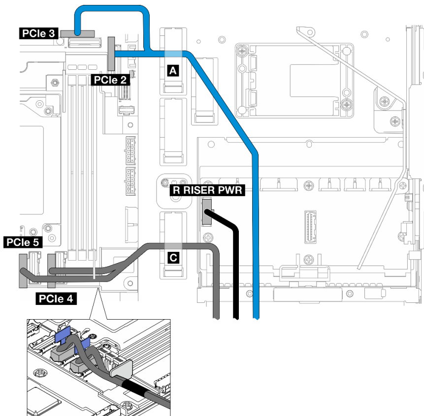
Abbildung 136. Kabelführung für PCIe-Adapterkarte 2
