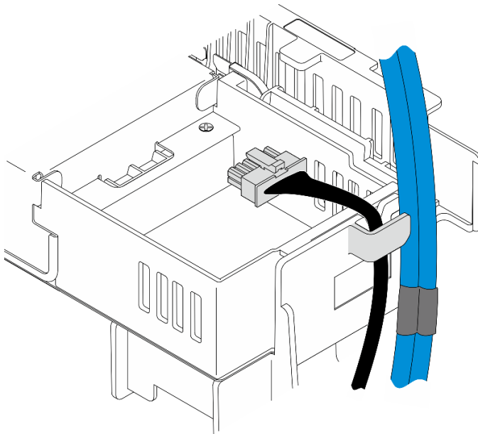
Abbildung 69. Interne Kabel der Rückwandplatine an der Kabelklemme
