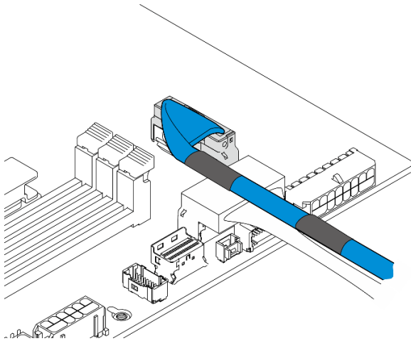
Abbildung 219. Internes BP-Signalkabel
