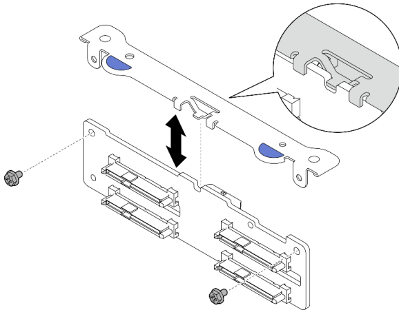
Abbildung 67. Trennen Sie die Rückwandplatine für Laufwerke von der Halterung für die Rückwandplatine
