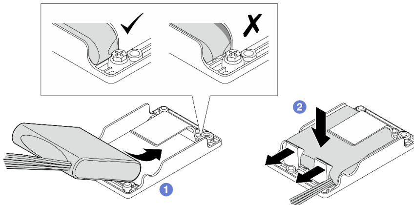
Abbildung 166. Installieren des RAID-Flash-Stromversorgungsmoduls
