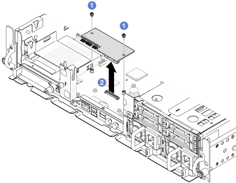
Abbildung 184. Entfernen des Firmware- und RoT-Sicherheitsmoduls
