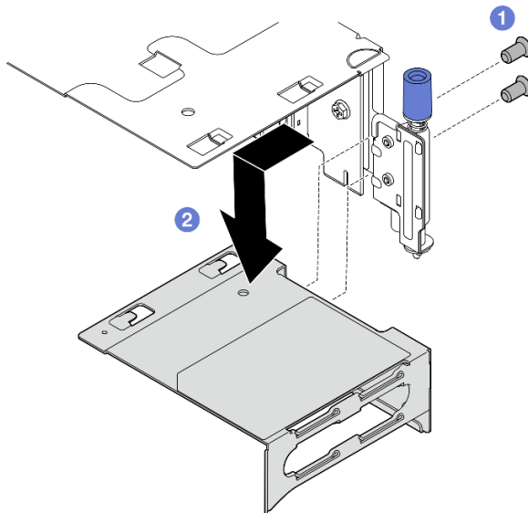
Abbildung 120. Extender aus PCIe-Adapterkarte 1 entfernen
