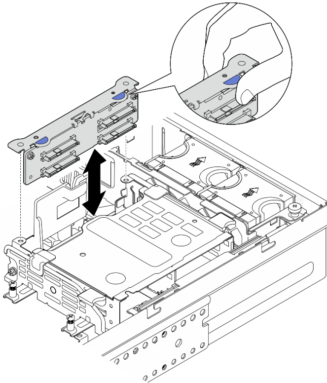
Abbildung 139. Interne Rückwandplatine für Laufwerke installieren
