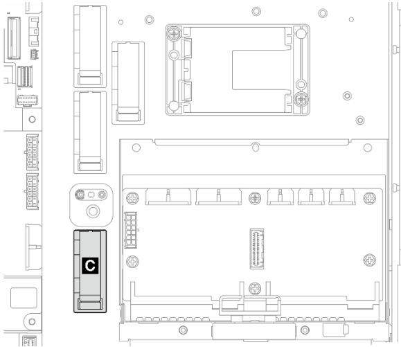
Abbildung 214. Kabelklemme C
