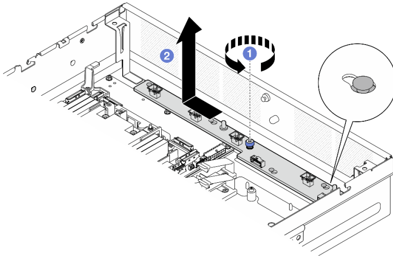
Abbildung 51. Lüfterplatine entfernen
