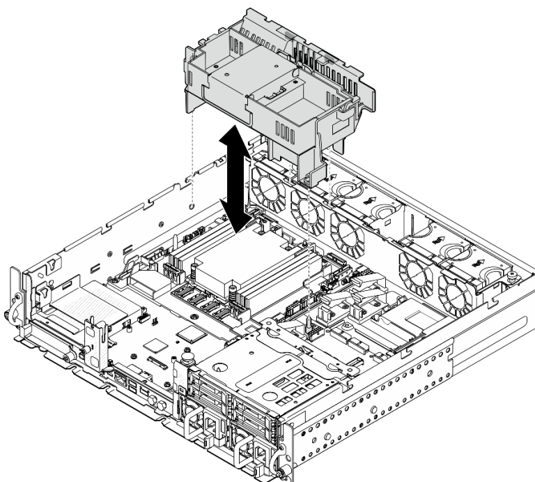
Abbildung 31. Luftführung für 1U-Kühlkörper entfernen
