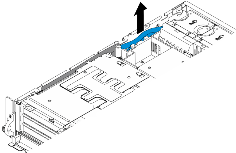
Abbildung 107. Signalkabel von PCIe-Adapter 1 lösen
