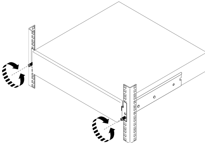
Abbildung 2. Trennen des Servers aus dem Rack: Standard-EIA-Halterungen
