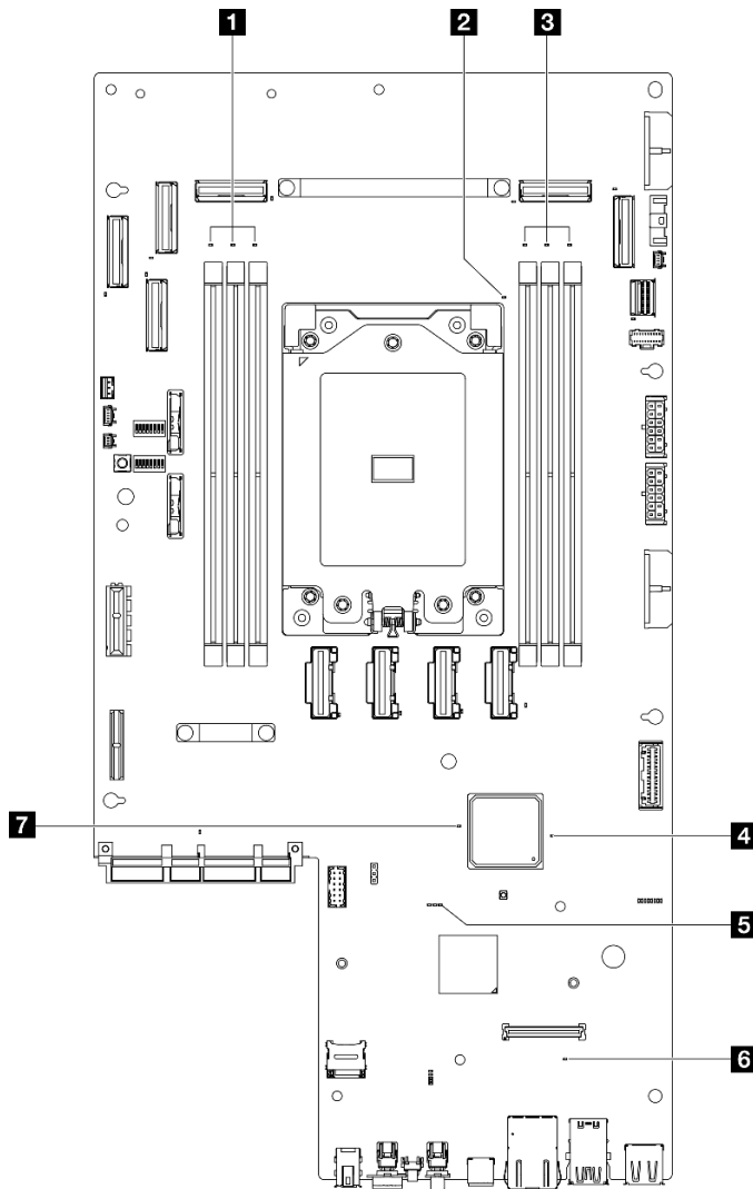
Abbildung 233. Anzeigen auf der Systemplatine
