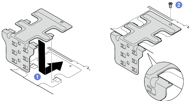
Abbildung 130. Seitliche Halterung installieren
