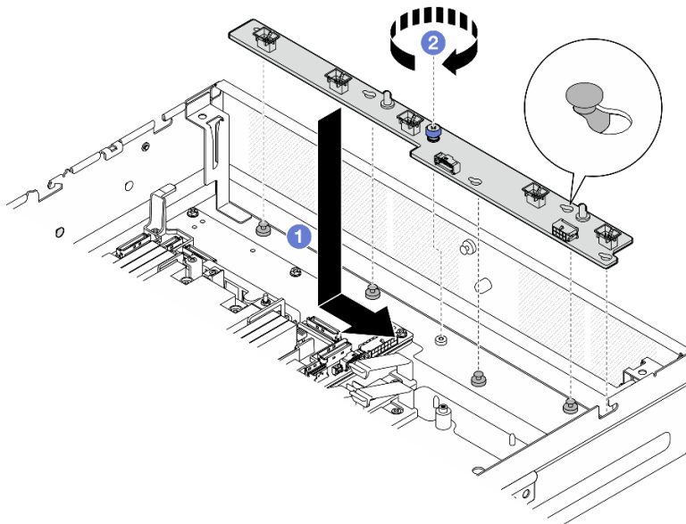
Abbildung 52. Lüfterplatine installieren
