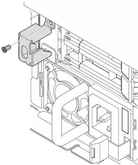
Abbildung 176. Schlüsselhalterung für Sicherheitsfrontblende entfernen
