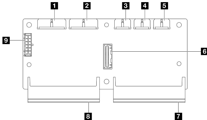
Abbildung 197. Anschlüsse für Stromversorgungsplatine
