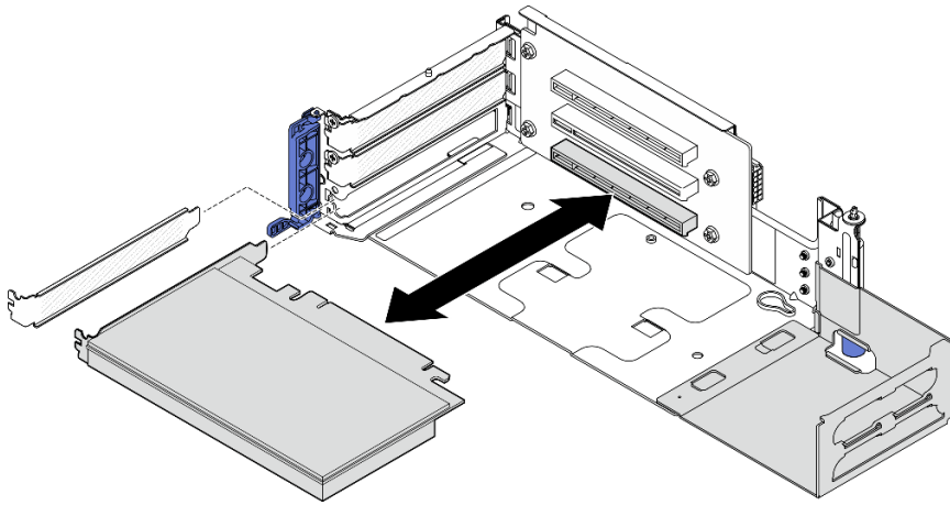
Abbildung 119. PCIe-Adapter aus PCIe-Adapterkarte 2 entfernen
