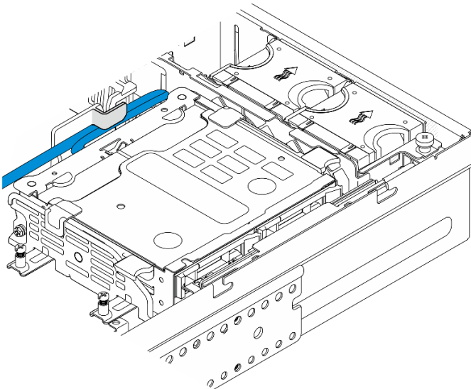
Abbildung 140. Kabelführung
