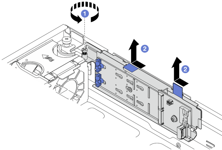
Abbildung 81. M.2-Rückwandplattenbaugruppe entfernen
