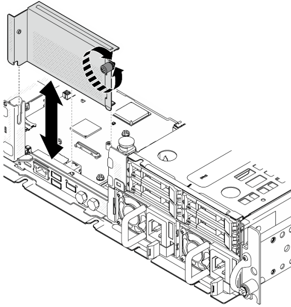
Abbildung 135. Entfernen der Abdeckblende für Adapterkarte
