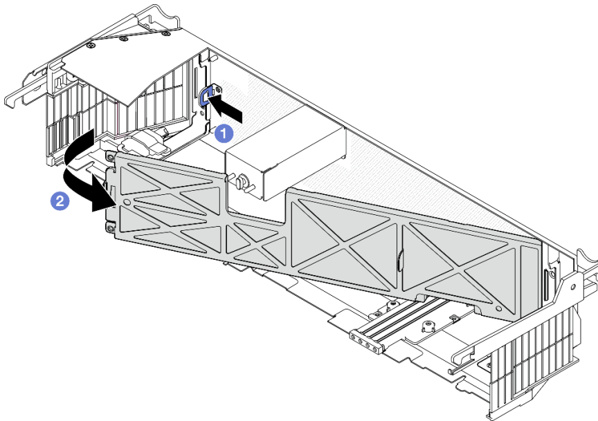
Abbildung 172. Entfernen des Staubfilters
