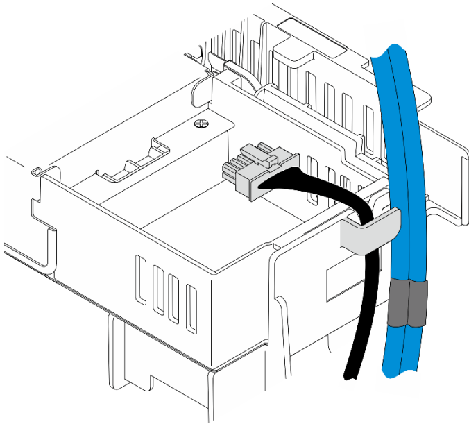
Abbildung 72. Interne Kabel der Rückwandplatine an der Kabelklemme
