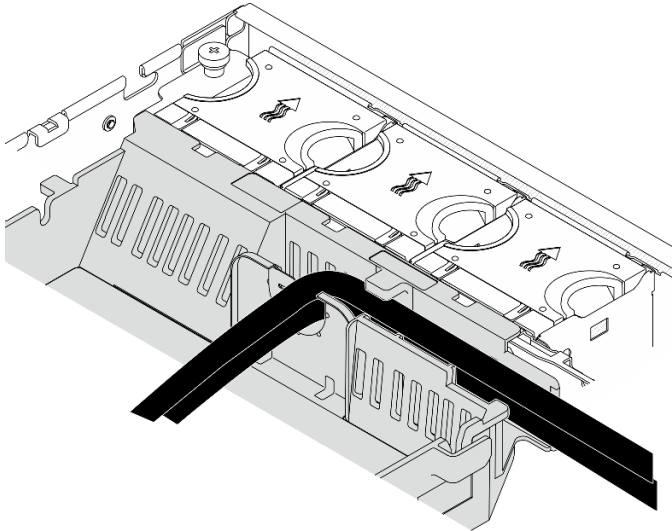
Abbildung 138. GPU-Netzkabel an der Prozessorluftführung
