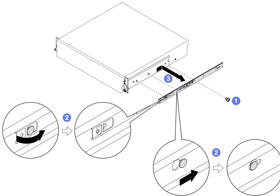
Abbildung 5. Inneren Schiene entfernen
