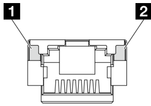
Abbildung 231. Anzeigen am XCC-Systemmanagementanschluss
