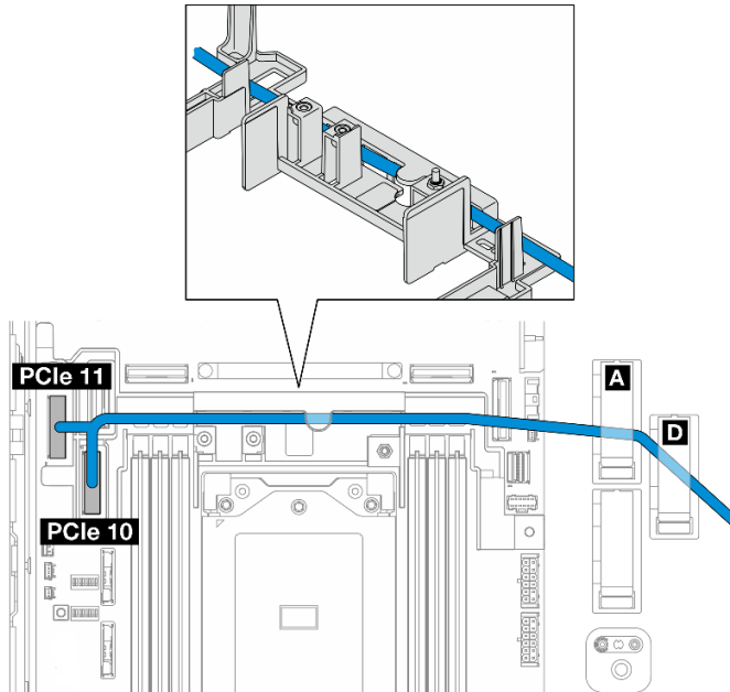
Abbildung 222. Vorderes BP-Signalkabel
