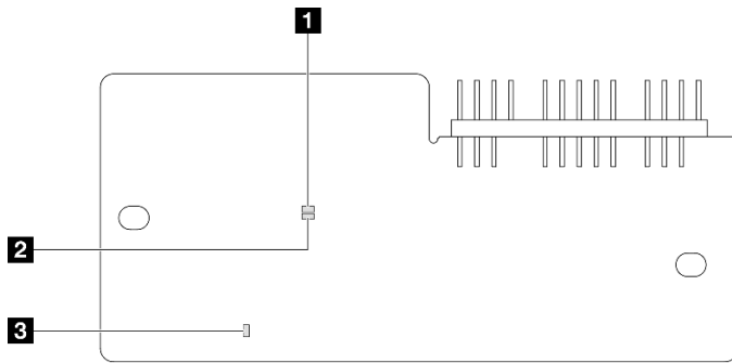
Abbildung 234. Anzeigen am Firmware- und RoT-Sicherheitsmodul
