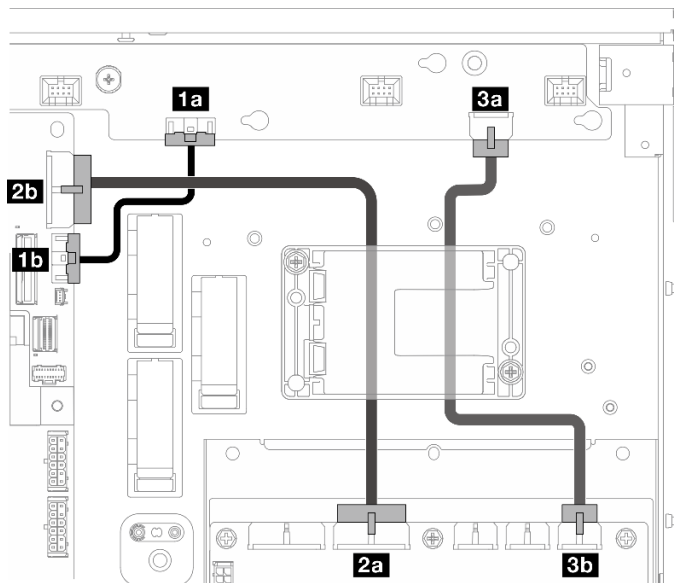
Abbildung 203. PDB- und FCB-Kabelführung
