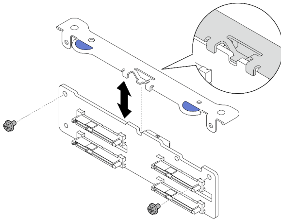
Abbildung 71. Rückwandplatine an der Rückwandplatinenhalterung sichern
