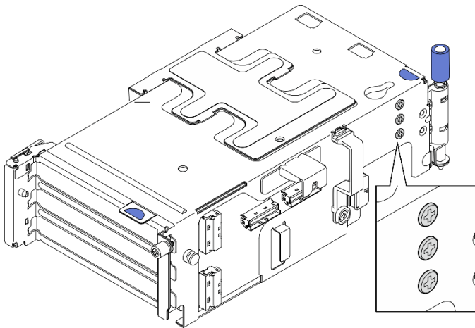
Abbildung 128. Ersatzschrauben am PCIe-Adapter 2
