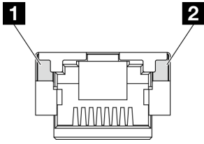
Abbildung 235. Anzeigen am XCC-Systemmanagementanschluss
