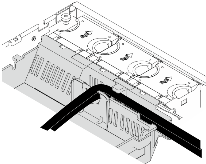
Abbildung 134. GPU-Netzkabel an der Prozessorluftführung
