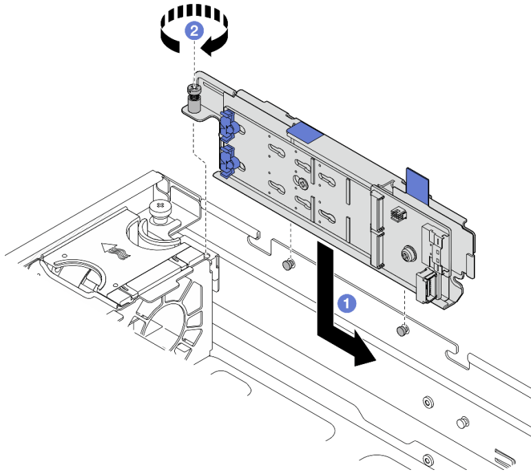
Abbildung 95. M.2-Rückwandplattenbaugruppe installieren
