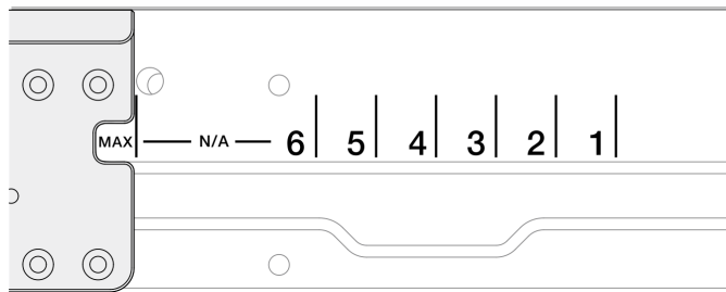
Abbildung 17. Tiefenmarkierung für EIA-Halterungen
