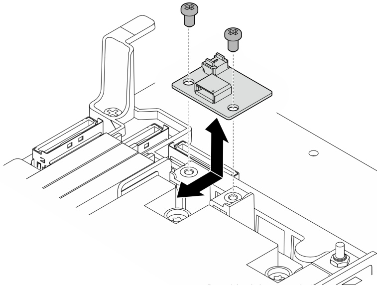
Abbildung 38. Entfernen der Luftmassensensorplatte
