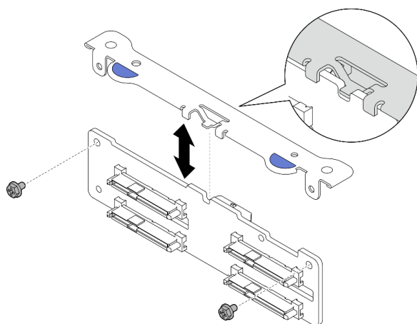
Abbildung 57. Trennen Sie die Rückwandplatte für Laufwerke von der Halterung für die Rückwandplatte
