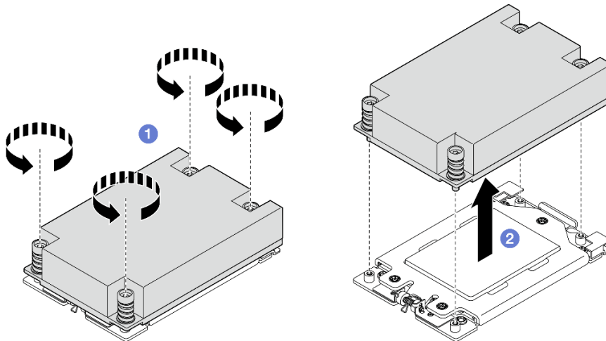
Abbildung 156. 1U-Kühlkörper entfernen
