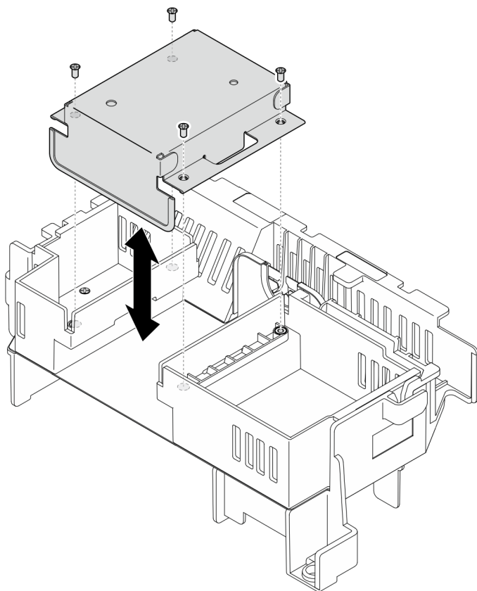
Abbildung 35. Mittlere Abdeckblende austauschen
