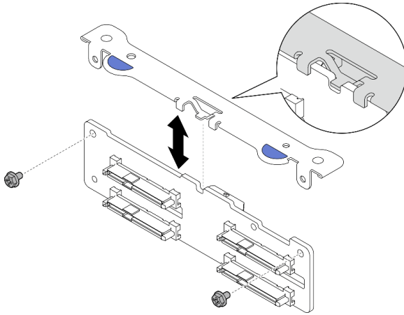
Abbildung 58. Rückwandplatine an der Rückwandplatinenhalterung sichern
