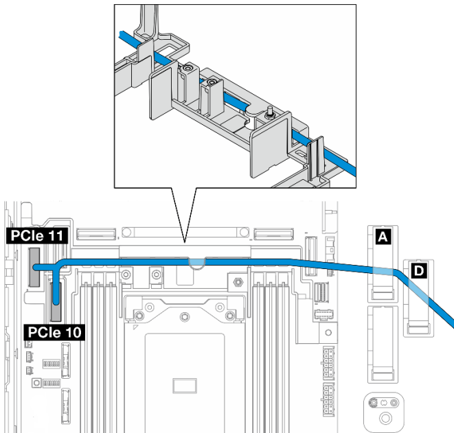
Abbildung 217. Vorderes BP-Signalkabel
