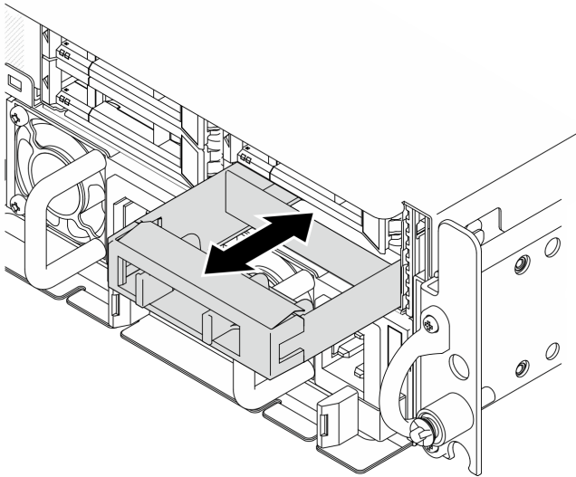
Abbildung 55. Installieren der Abdeckblende für Laufwerke
