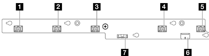
Abbildung 196. Anschlüsse Lüfterplatine
