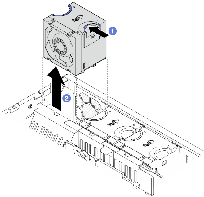
Abbildung 48. Entfernen eines Lüftermoduls
