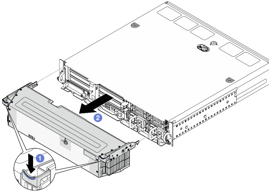
Abbildung 171. Entfernen der Sicherheitsfrontblende
