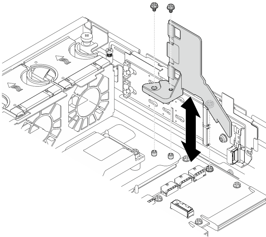
Abbildung 25. M.2-Luftführung für eine Konfiguration mit interner Laufwerkhalterung entfernen
