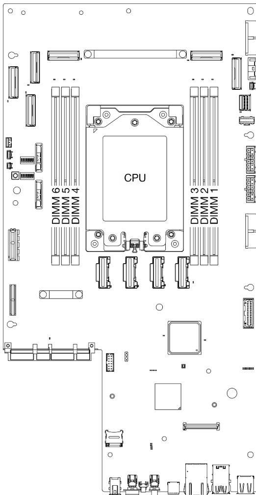
Abbildung 98. Layout für Speichermodule und Prozessor
