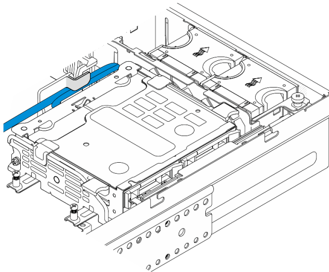
Abbildung 74. Kabelführung der internen Rückwandplatine für Laufwerke
