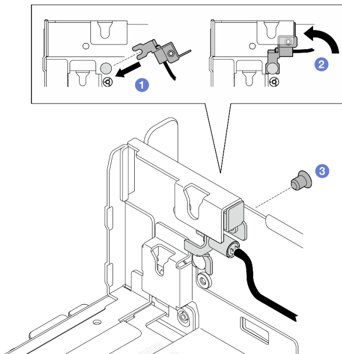
Abbildung 41. Frontblendenerkennungsschalter installieren
