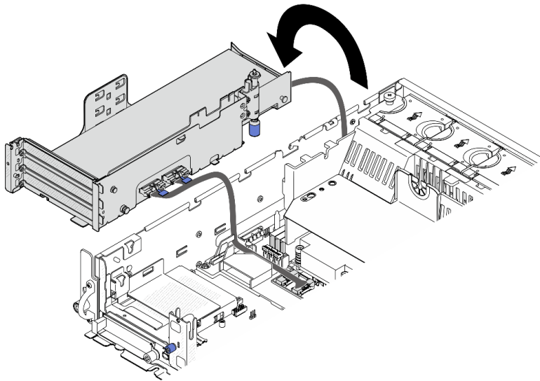
Abbildung 109. PCIe-Adapter 1 neben dem Gehäuse platzieren
