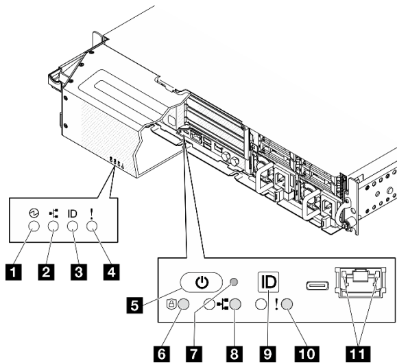
Abbildung 230. Anzeigen an der Vorderseite
