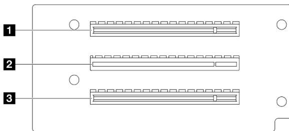
Abbildung 201. PCIe-Adapterkarte 2
