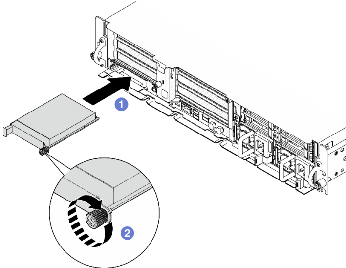
Abbildung 105. Installieren des OCP-Moduls
