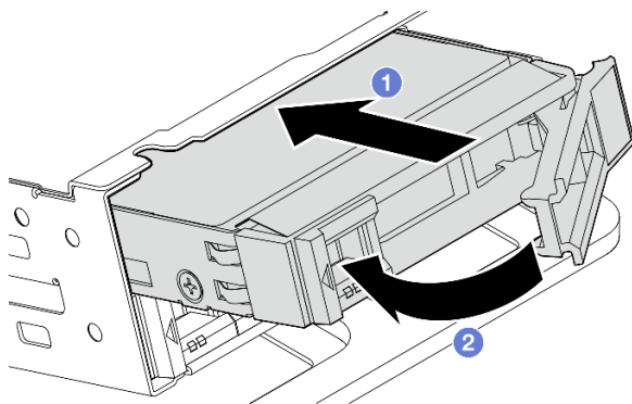
Abbildung 77. Internes Laufwerk installieren
