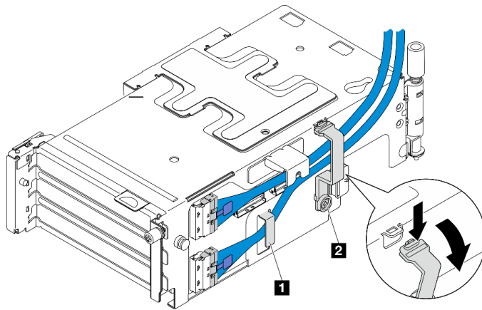
Abbildung 141. Kabelführung für PCIe-Adapterkarte 2
