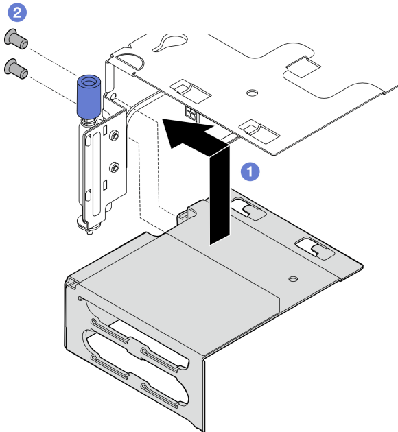
Abbildung 123. Erweiterung für PCIe-Adapter 2 installieren
