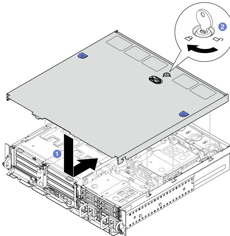
Abbildung 193. Installieren der oberen Abdeckung
