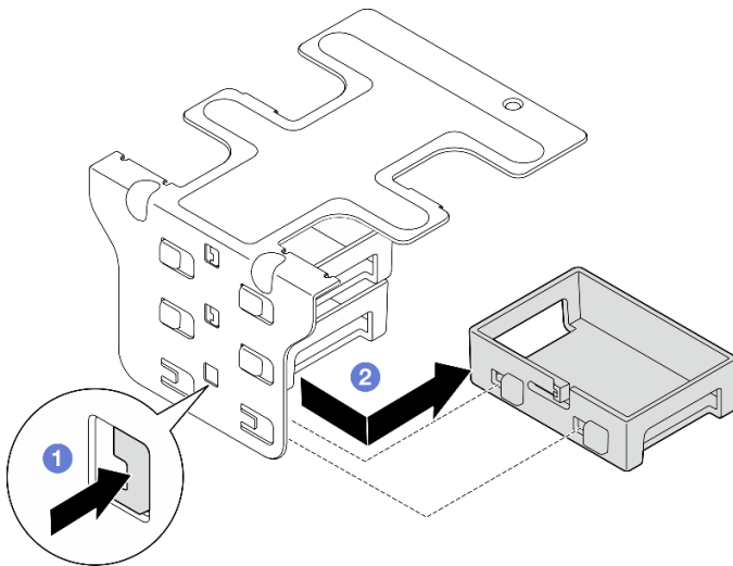
Abbildung 116. Flache Abdeckblende entfernen
