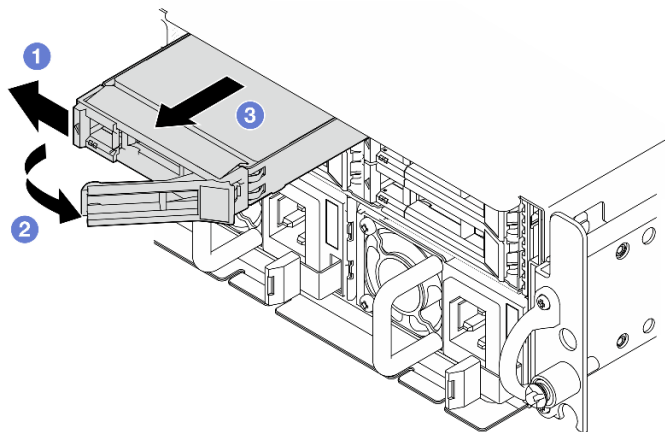
Abbildung 54. Vorderes Hot-Swap-Laufwerk entfernen
