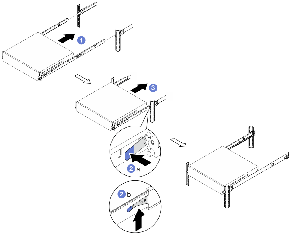
Abbildung 22. Server im Rack installieren
