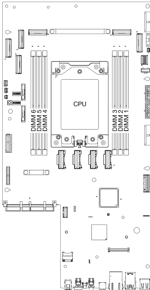
Abbildung 96. Layout für Speichermodule und Prozessor
