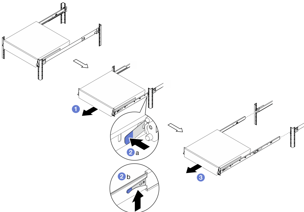
Abbildung 4. Server aus dem Rack entfernen
