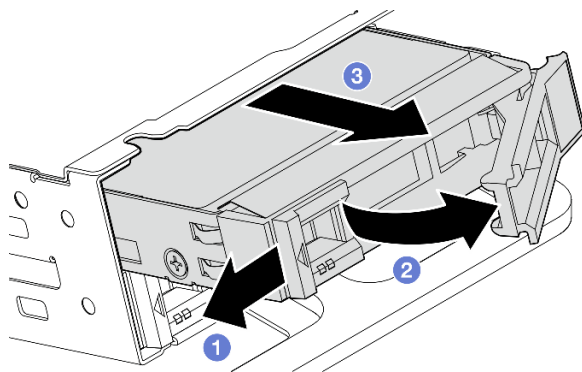
Abbildung 64. Internes Laufwerk entfernen
