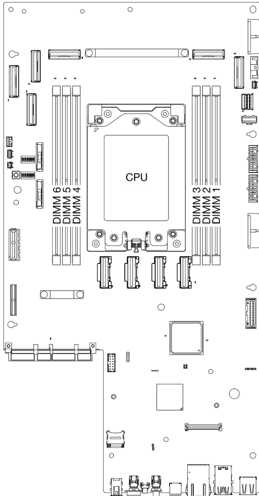
Abbildung 1. Layout für Speichermodule und Prozessor
