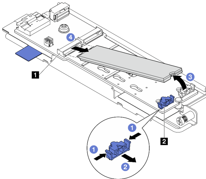
Abbildung 85. Entfernen eines M.2-Laufwerks
