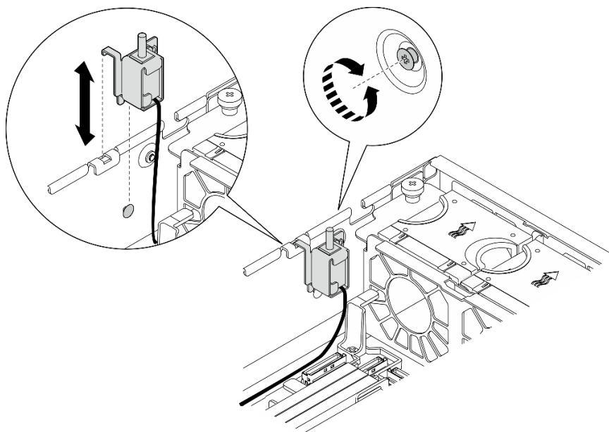
Abbildung 79. Entfernen des Schalters gegen unbefugten Zugriff mit Kabel
