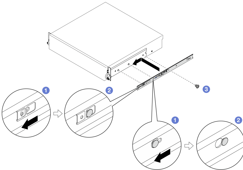
Abbildung 16. Inneren Schiene installieren
