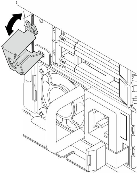
Abbildung 178. Halterung für Schlüsselhalterung für Sicherheitsfrontblende installieren
