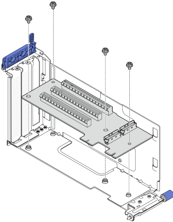
Abbildung 144. Installieren der Adapterkarte
