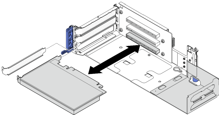
Abbildung 125. PCIe-Adapter in PCIe-Adapterkarte 2 installieren
