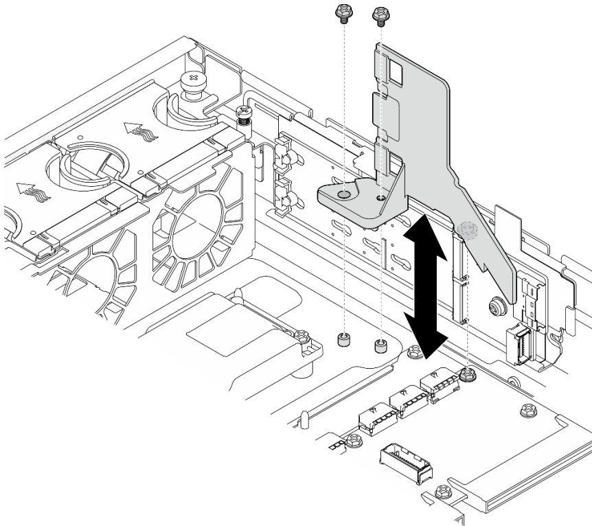
Abbildung 29. M.2-Luftführung für eine Konfiguration mit interner Laufwerkhalterung installieren
