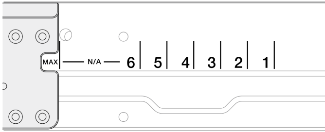
Abbildung 13. Tiefenmarkierung für EIA-Halterungen
