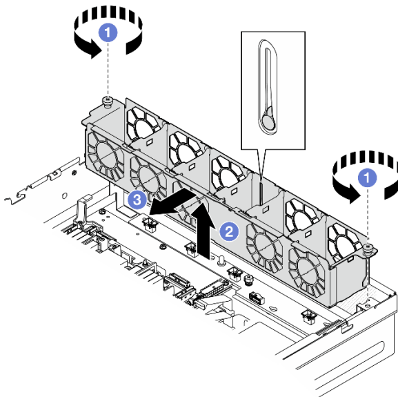
Abbildung 50. Lüfterrahmen entfernen
