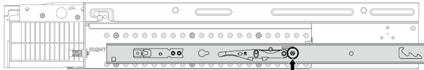
Abbildung 7. Eine Schraube für die innere Schiene des ThinkEdge Kugellager-Schienenatz für 600-mm-Rack
