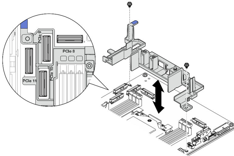
Abbildung 42. Kabelwand entfernen
