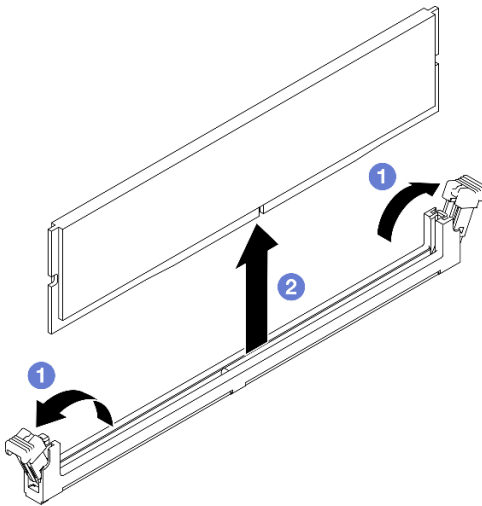
Abbildung 97. Speichermodul entfernen
