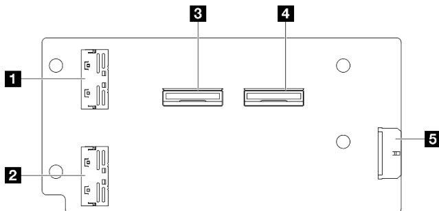
Abbildung 200. PCIe-Adapterkarte 2
