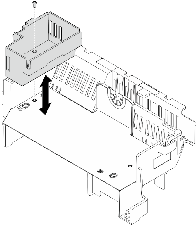
Abbildung 33. Abdeckblende für die Adapterkarte 1 austauschen
