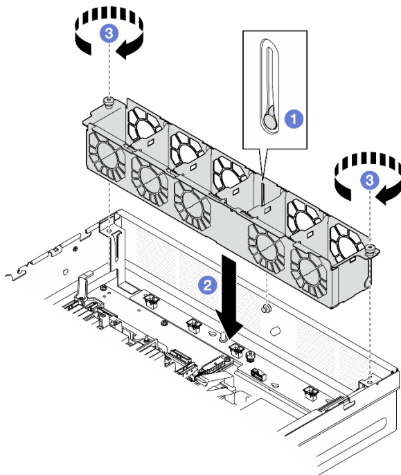
Abbildung 53. Installieren des Systemlüfterrahmens
