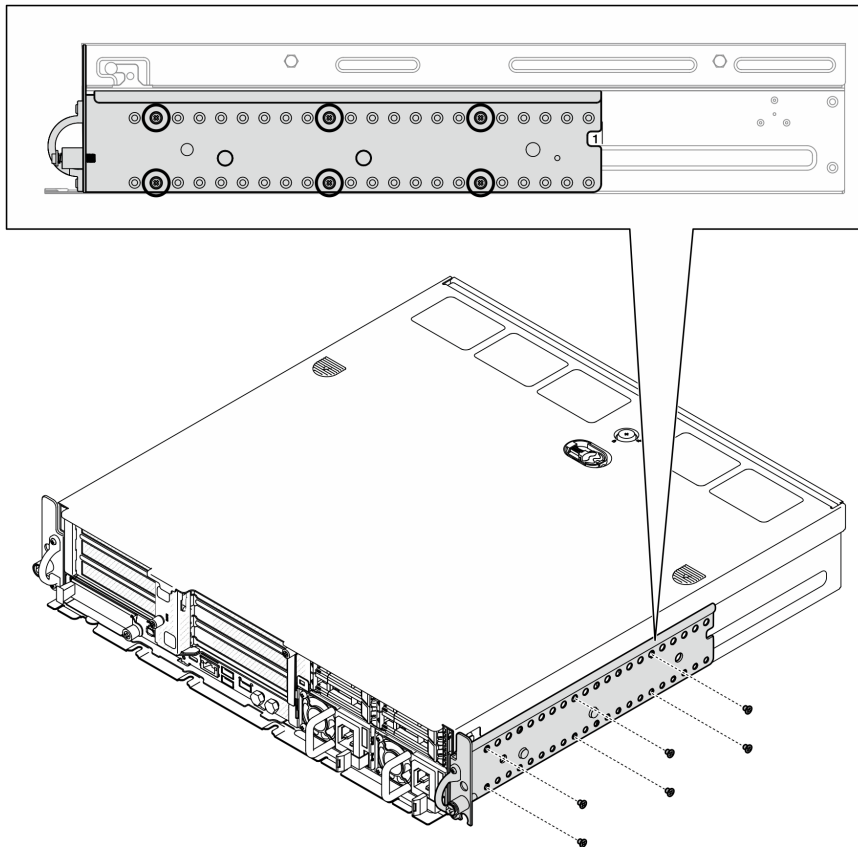
Abbildung 11. EIA-Halterung mit normaler Tiefe 1 bis 6: sechs Schrauben
