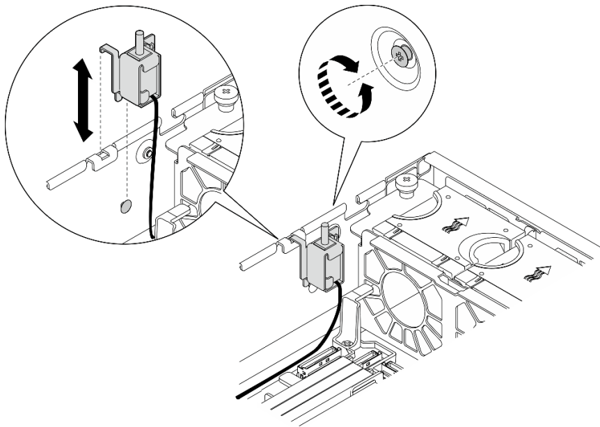
Abbildung 80. Installieren des Schalters gegen unbefugten Zugriff
