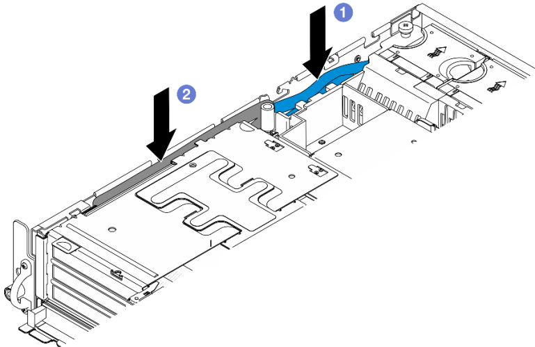
Abbildung 133. Signalkabel für PCIe-Adapter 1 verlegen
