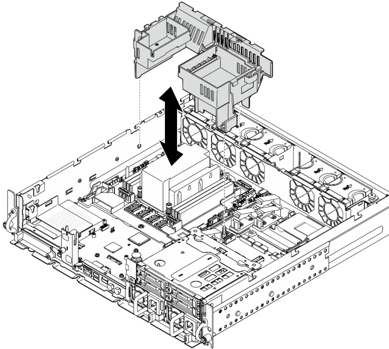
Abbildung 32. Luftführung für 2U-Kühlkörper entfernen
