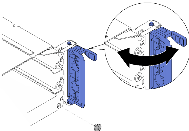
Abbildung 183. Unverlierbare Schrauben installieren
