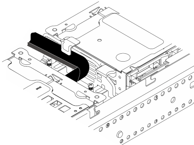
Abbildung 75. Kabelführung der vorderen Rückwandplatine für Laufwerke
