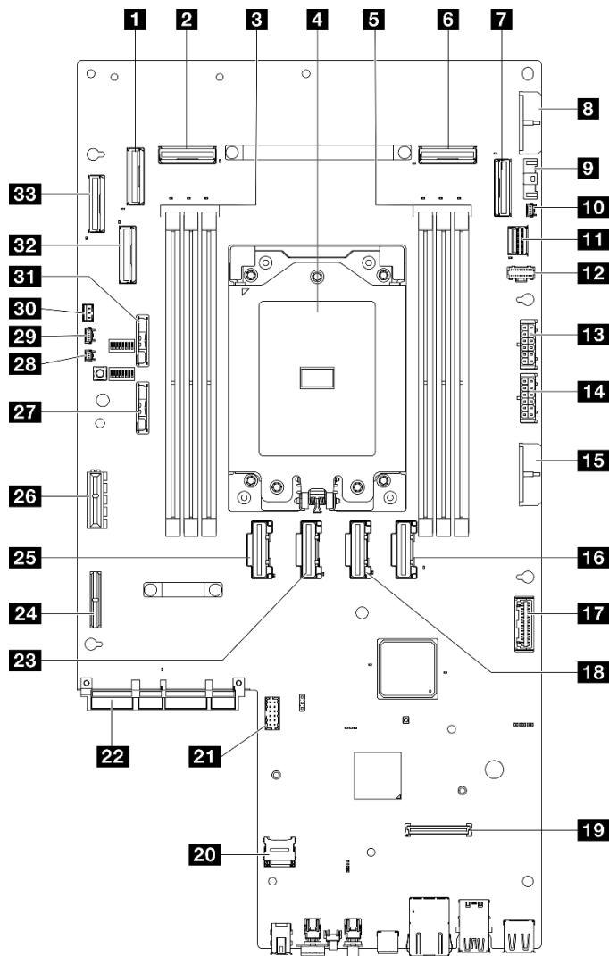
Abbildung 228. Anschlüsse auf der Systemplatine
