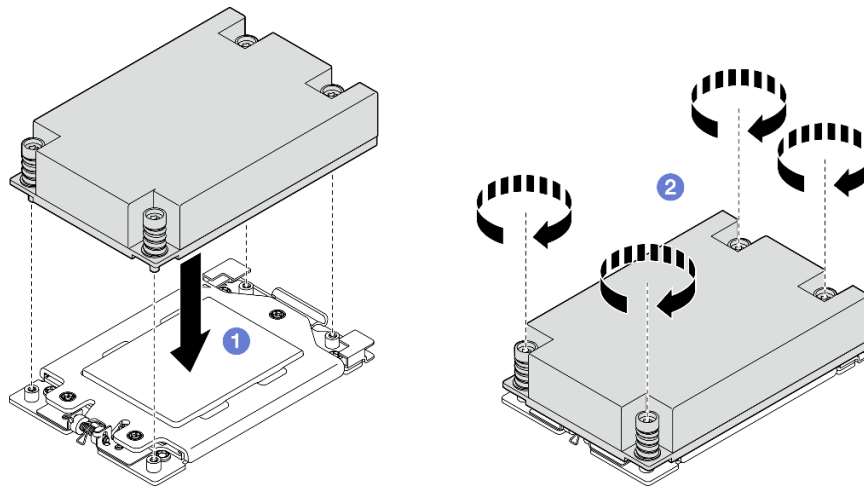
Abbildung 161. 1U-Kühlkörper installieren
