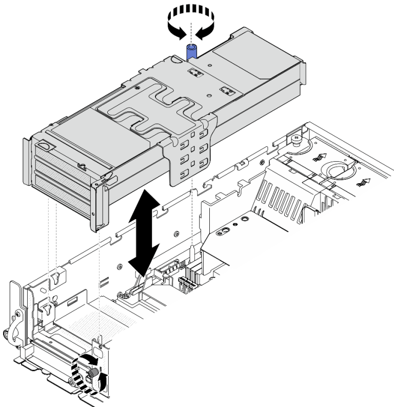
Abbildung 108. PCIe-Adapterkarte 1 hochheben
