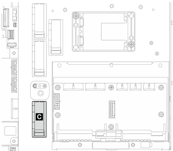
Abbildung 223. Kabelklemme C
