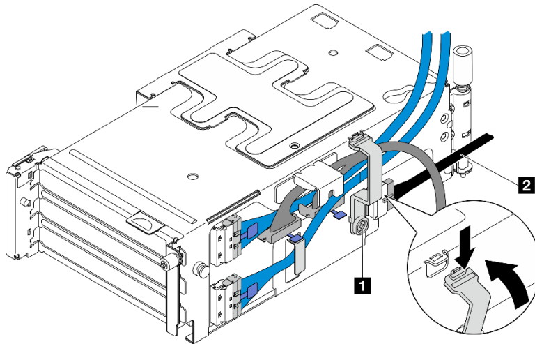
Abbildung 149. Kabelführung für PCIe-Adapterkarte 2
