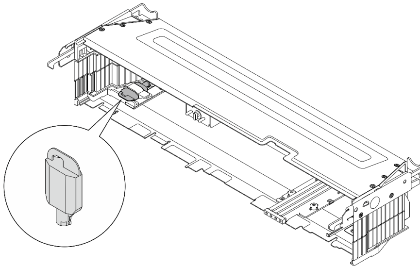
Abbildung 174. Aufbewahrungsort des Schlüssels für die Sicherheitsfrontblende
