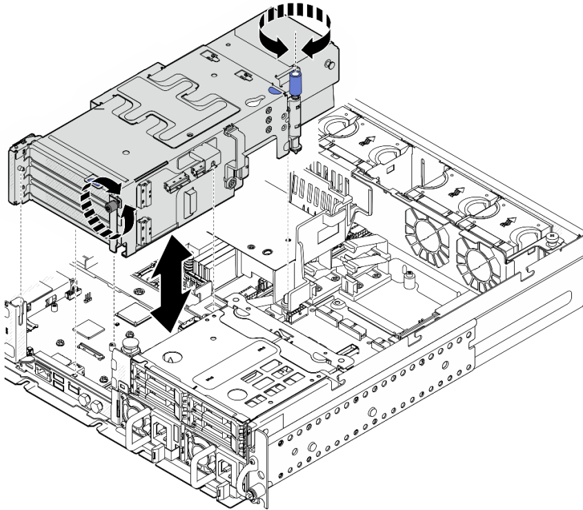
Abbildung 137. Installieren von PCIe-Adapterkarte 2
