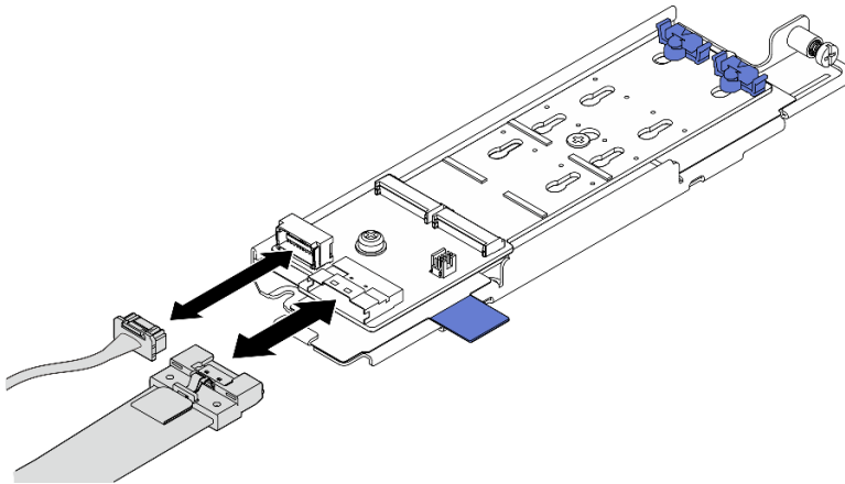
Abbildung 93. Verbinden des Kabels zur SATA/x4 NVMe-M.2-Rückwandplatine
