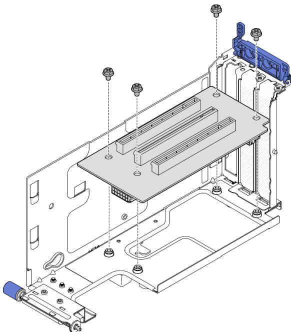
Abbildung 143. Adapterkarte von PCIe-Adapterkarte 2 entfernen
