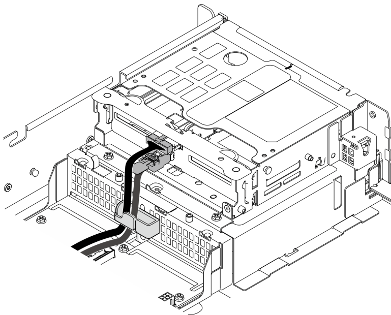
Abbildung 60. Kabelführung der vorderen Rückwandplatine für Laufwerke
