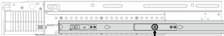
Abbildung 19. Eine Schraube für die innere Schiene der ThinkEdge 2-Pfosten-Reibungsschienensatz
