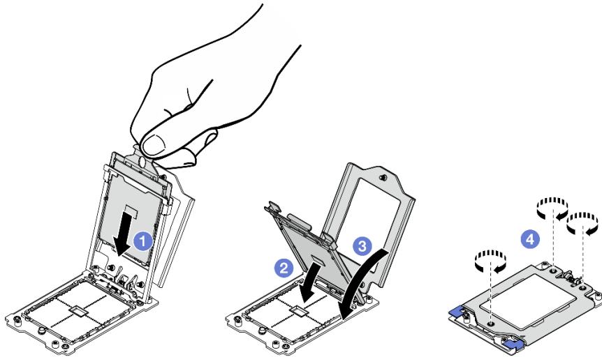
Abbildung 159. Installieren eines Prozessors
