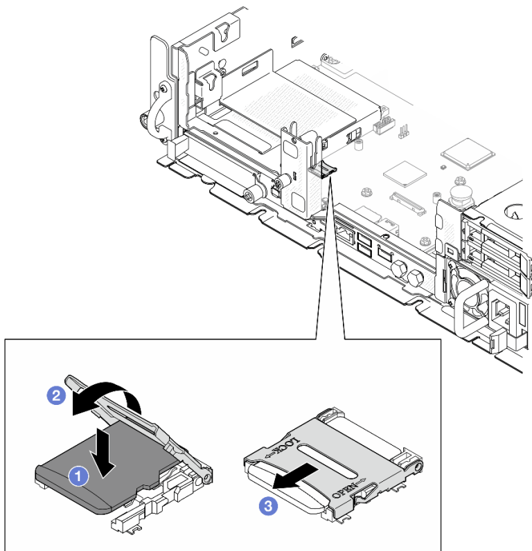
Abbildung 101. Installieren der microSD-Karte
