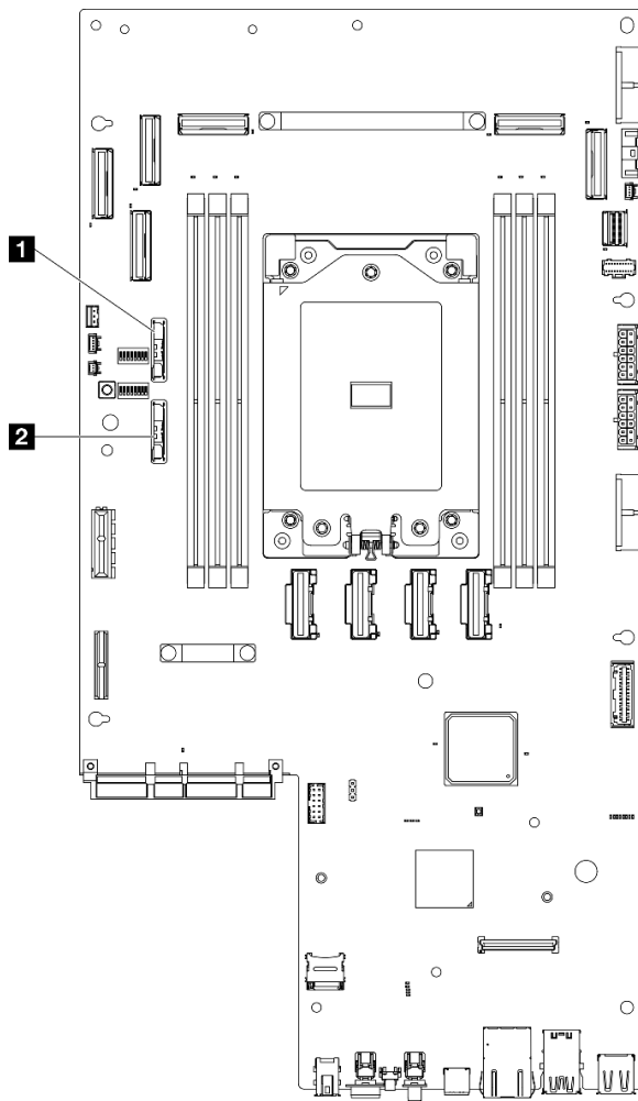
Abbildung 44. Positionen der CMOS-Batterie auf der Systemplatine
