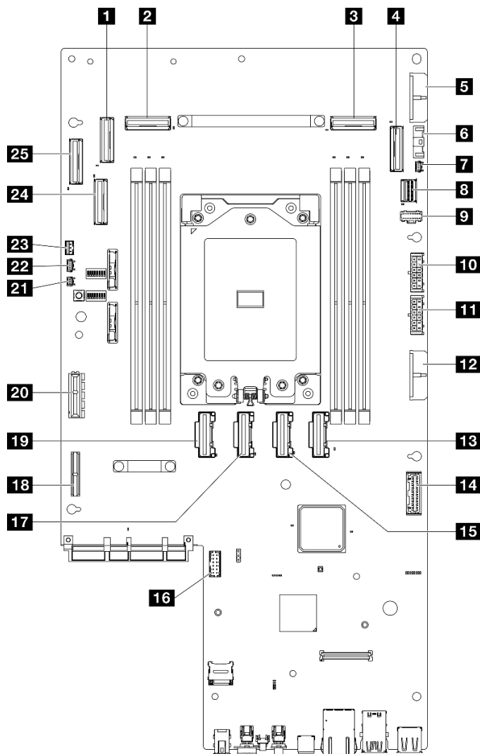
Abbildung 202. Anschlüsse auf der Systemplatine
