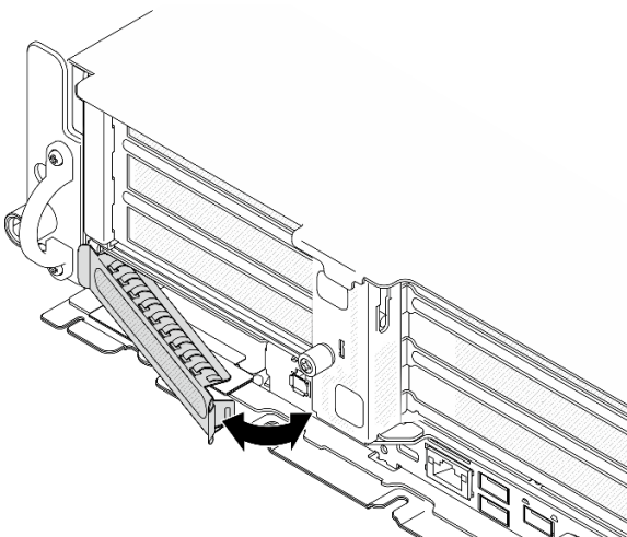
Abbildung 103. OCP-Abdeckblende installieren
