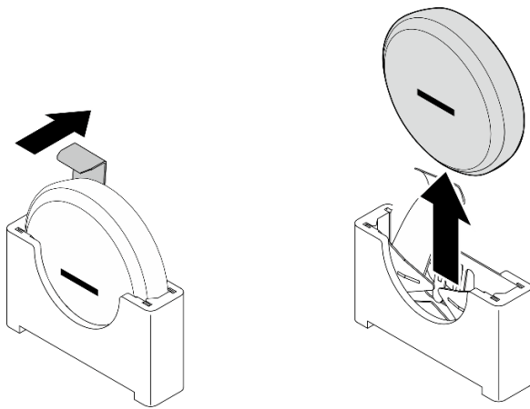
Abbildung 45. Entfernen der CMOS-Batterie
