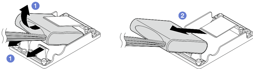
Abbildung 163. Entfernen des RAID-Flash-Stromversorgungsmoduls
