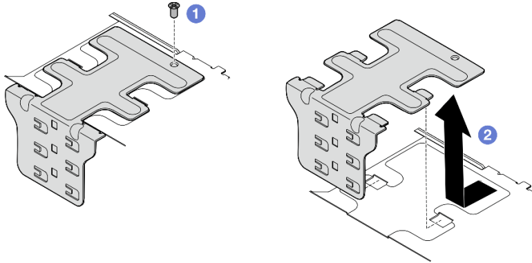
Abbildung 115. Seitliche Halterung entfernen
