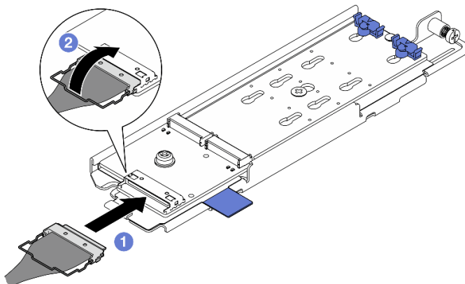
Abbildung 94. Verbinden des Kabels zur SATA/NVMe-M.2-Rückwandplatine
