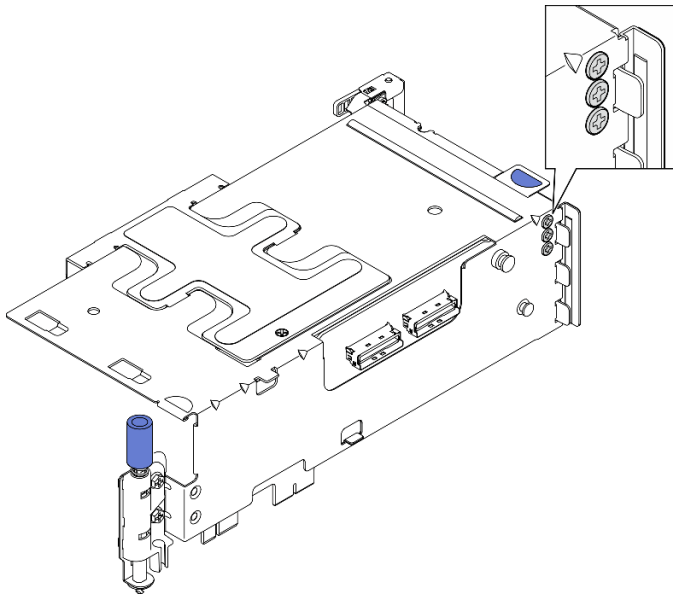
Abbildung 127. Ersatzschrauben am PCIe-Adapter 1
