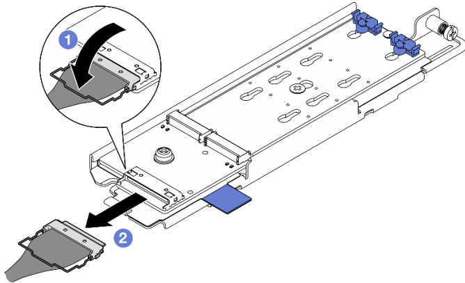
Abbildung 83. Abziehen des Kabels von der SATA/NVMe-M.2-Rückwandplatine
