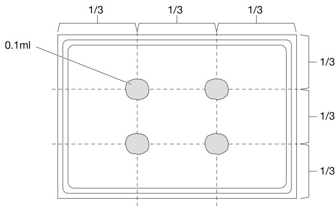
Abbildung 160. Auftragen der Wärmeleitpaste
