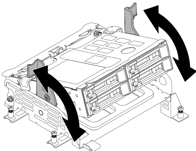
Abbildung 78. Interne Laufwerkhalterung drehen
