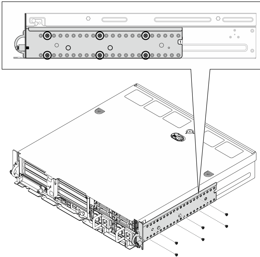
Abbildung 14. EIA-Halterung mit normaler Tiefe 1 bis 6: sechs Schrauben
