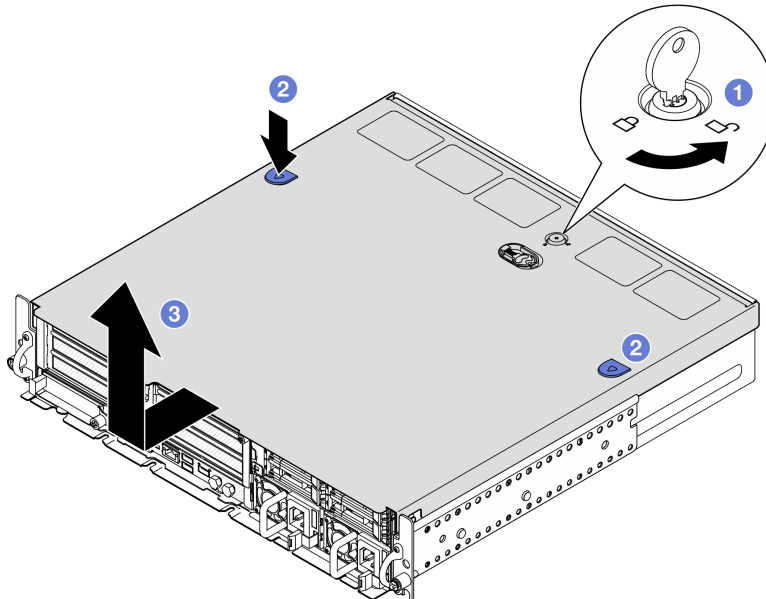
Abbildung 192. Entfernen der oberen Abdeckung
