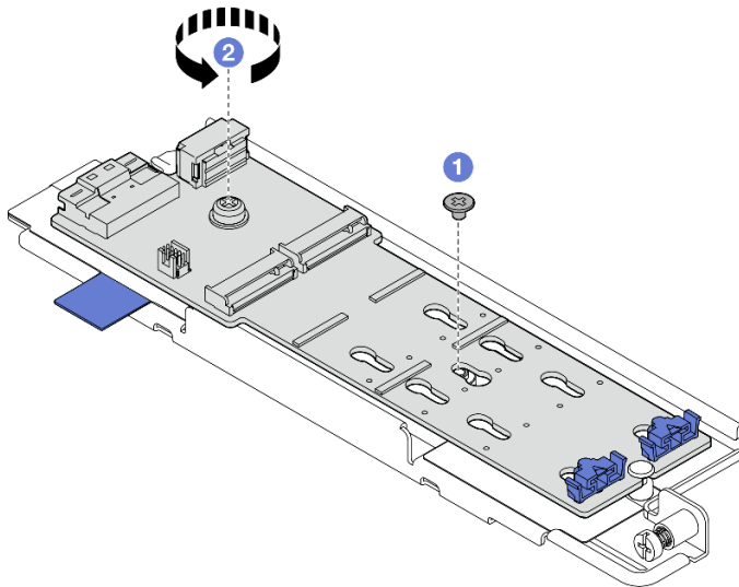
Abbildung 86. M.2-Rückwandplatine entfernen
