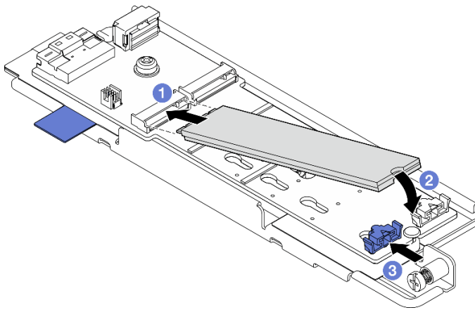
Abbildung 92. Installieren eines M.2-Laufwerks
