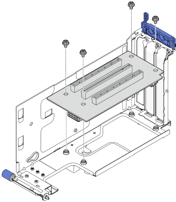
Abbildung 147. Installieren der Adapterkarte
