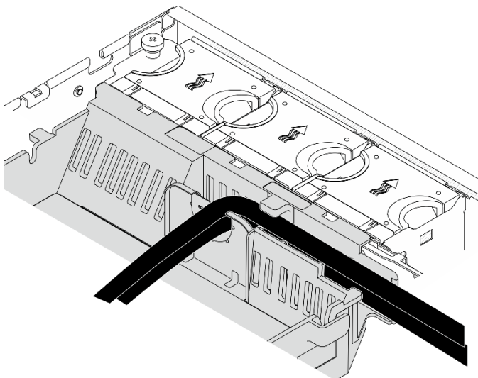
Abbildung 106. GPU-Netzkabel an der Prozessorluftführung
