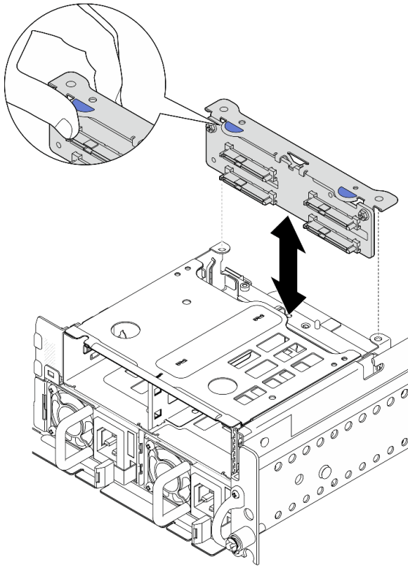
Abbildung 59. Vordere Rückwandplatine für Laufwerke installieren
