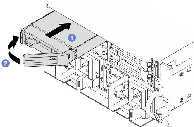
Abbildung 62. Vorderes Hot-Swap-Laufwerk installieren
