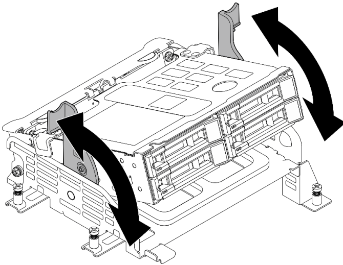
Abbildung 63. Interne Laufwerkhalterung drehen
