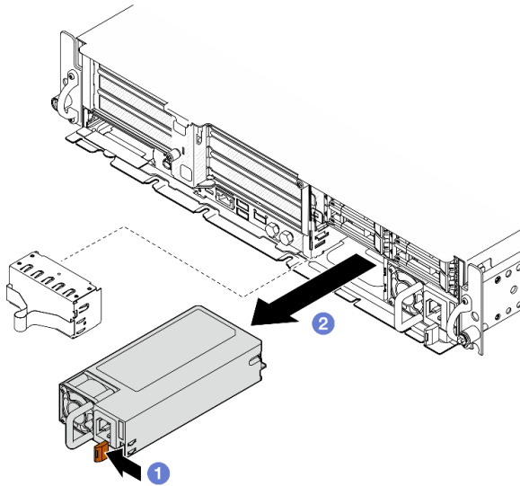
Abbildung 154. Entfernen der Netzteilereinheit
