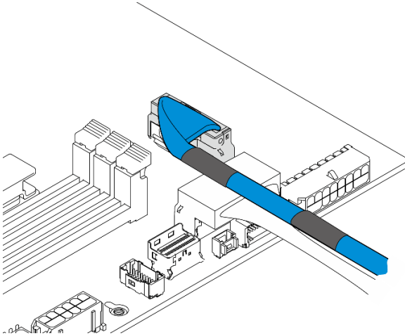
Abbildung 216. Internes BP-Signalkabel
