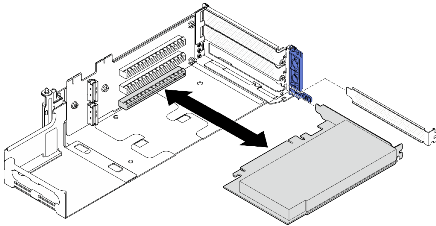
Abbildung 124. PCIe-Adapter in PCIe-Adapterkarte 1 installieren
