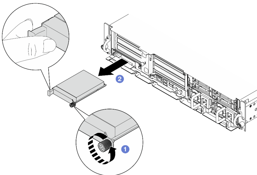
Abbildung 102. Herausnehmen des OCP-Moduls
