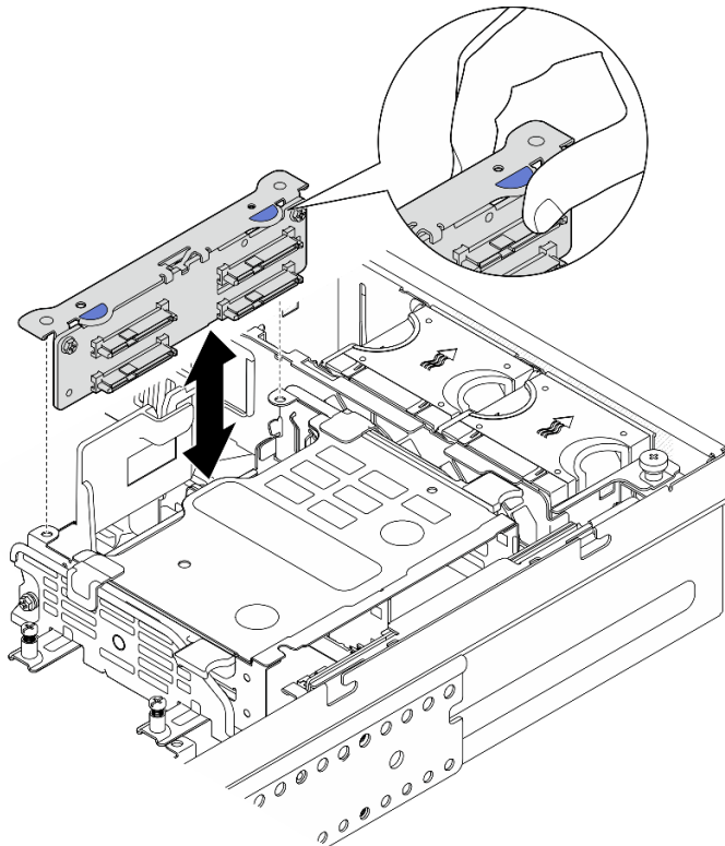
Abbildung 73. Interne Rückwandplatine für Laufwerke installieren
