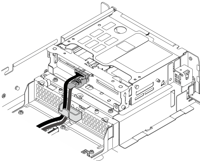
Abbildung 224. Kabelführung der vorderen Rückwandplatine für Laufwerke
