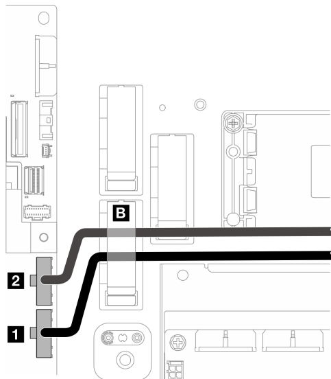
Abbildung 213. BP-Netzkabel
