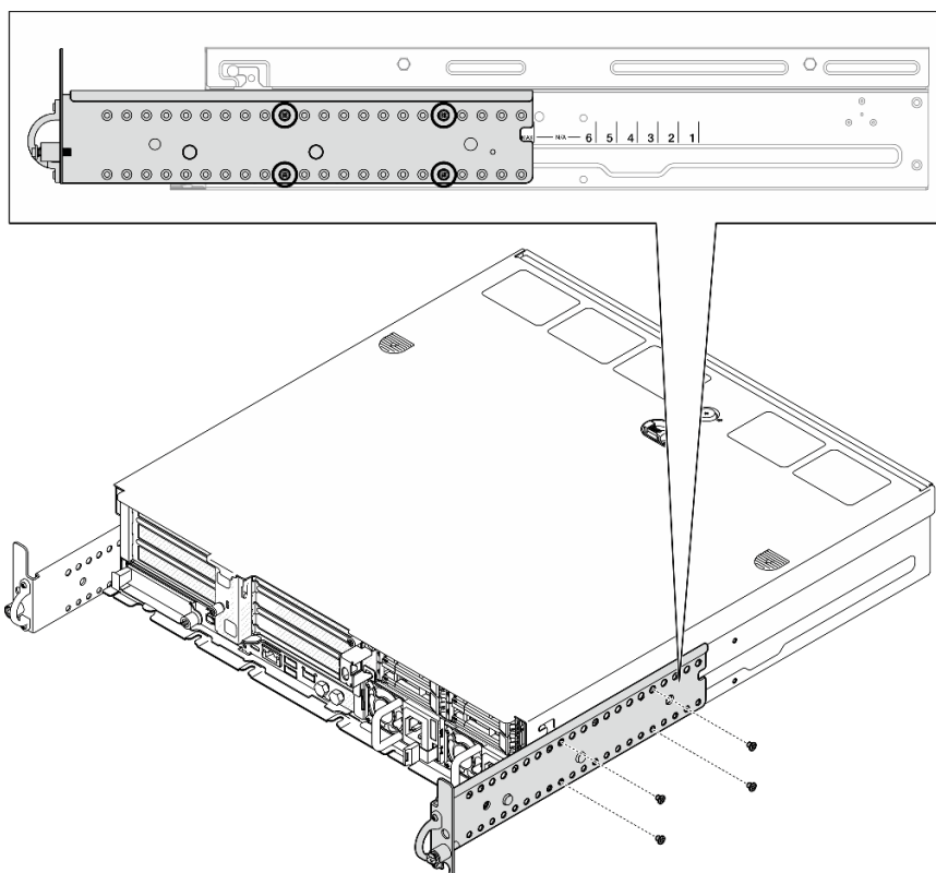
Abbildung 12. EIA-Halterung mit maximaler Tiefe für Sicherheitsfrontblende: vier Schrauben
