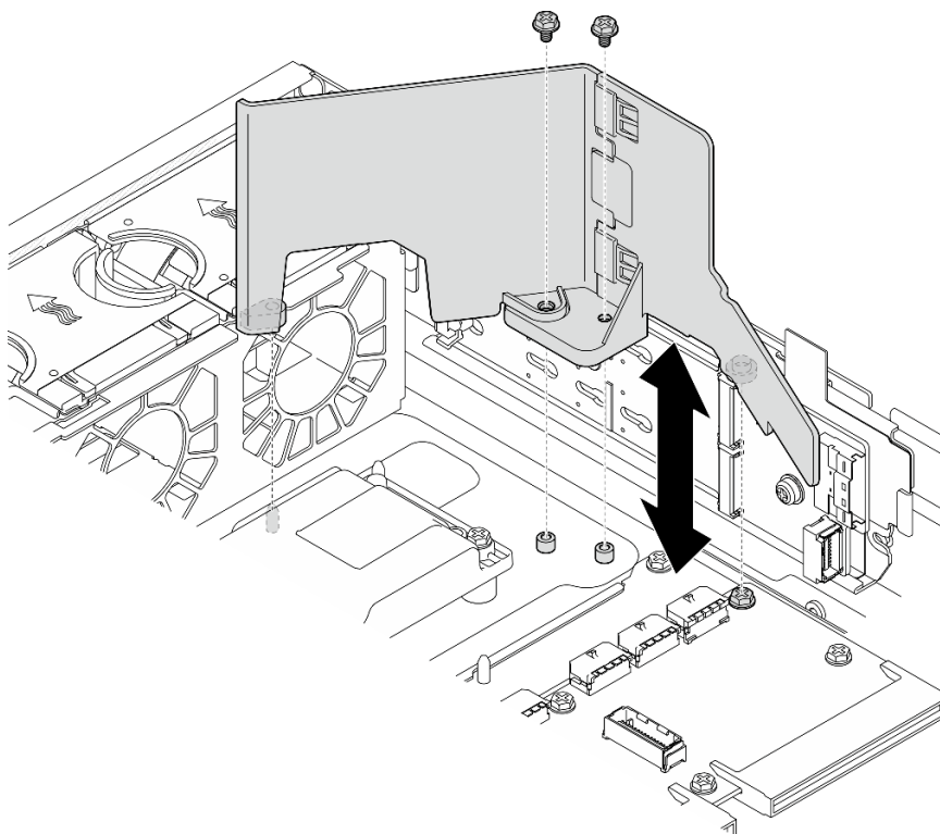
Abbildung 30. M.2-Luftführung für eine Konfiguration ohne interne Laufwerkhalterung installieren
