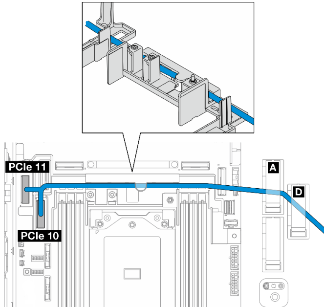
Abbildung 220. Vorderes BP-Signalkabel
