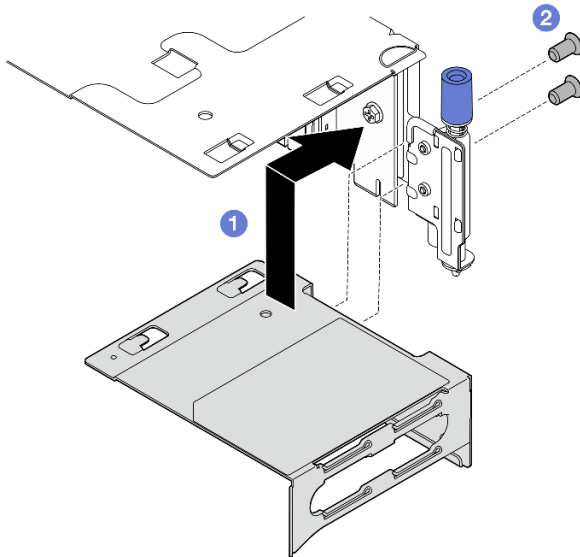
Abbildung 122. Erweiterung für den PCIe-Adapter 1 installieren
