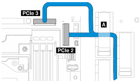
Abbildung 215. Internes BP-Signalkabel
