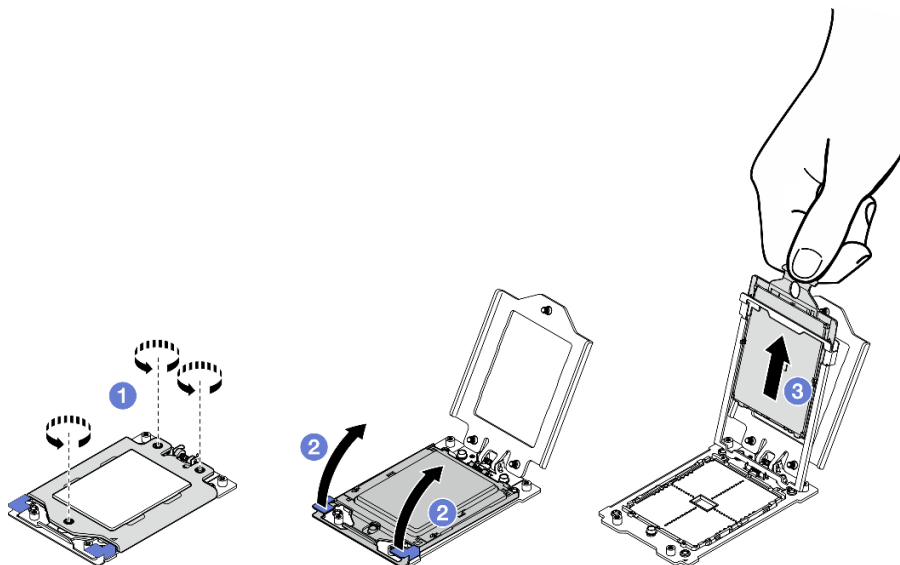
Abbildung 158. Entfernen eines Prozessors
