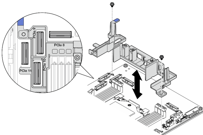
Abbildung 43. Kabelwand installieren
