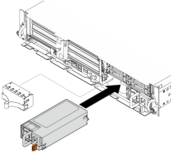
Abbildung 155. Installieren einer Netzteilereinheit
