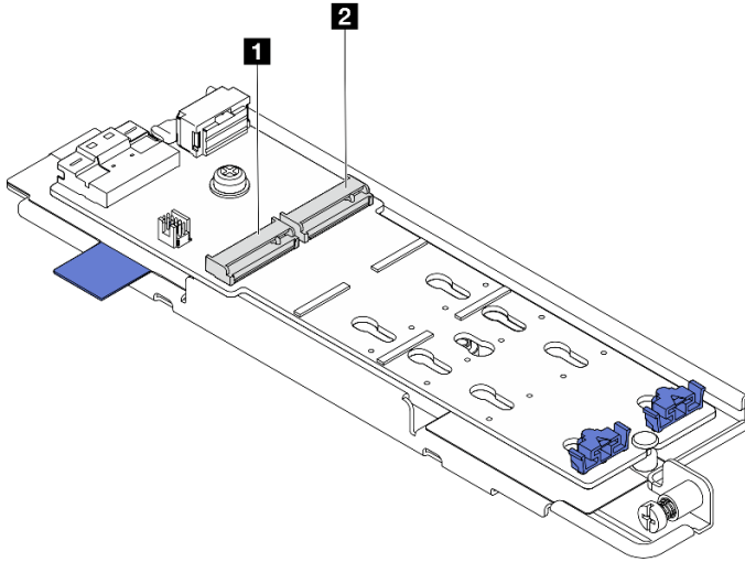
Abbildung 91. Steckplatznummerierung von M.2-Laufwerk
