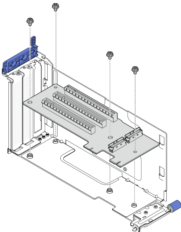
Abbildung 142. Adapterkarte von PCIe-Adapterkarte 1 entfernen
