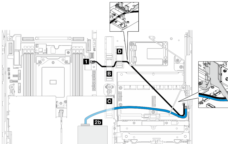
Abbildung 207. RAID-Adapter auf PCIe-Adapterkarte 2
