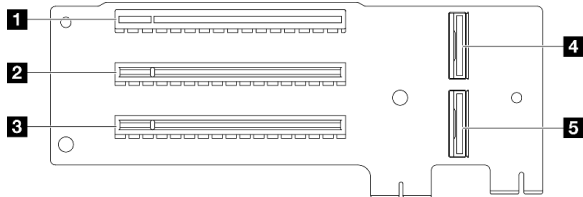
Abbildung 199. PCIe-Adapterkarte 1
