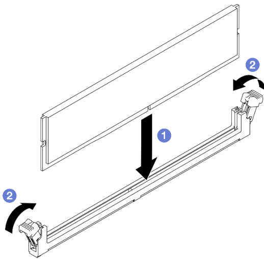
Abbildung 99. Installieren eines Speichermoduls
