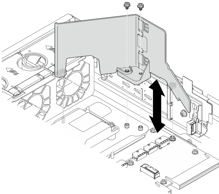
Abbildung 26. M.2-Luftführung für eine Konfiguration ohne interne Laufwerkhalterung entfernen
