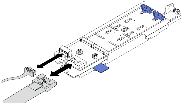
Abbildung 82. Abziehen des Kabels von der SATA/x4-NVMe-M.2-Rückwandplatine
