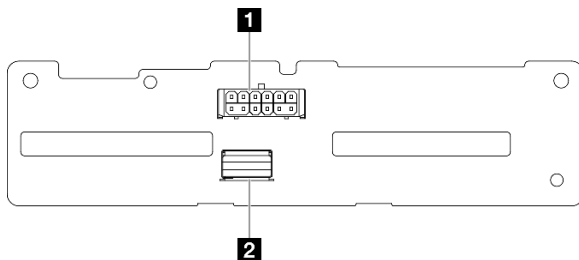
Abbildung 194. Anschlüsse auf der SAS/SATA-Rückwandplatine
