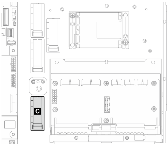
Abbildung 221. Kabelklemme C
