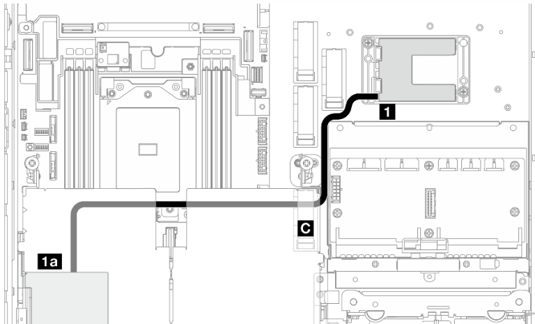
Abbildung 211. RAID-Adapter auf PCIe-Adapterkarte 1
