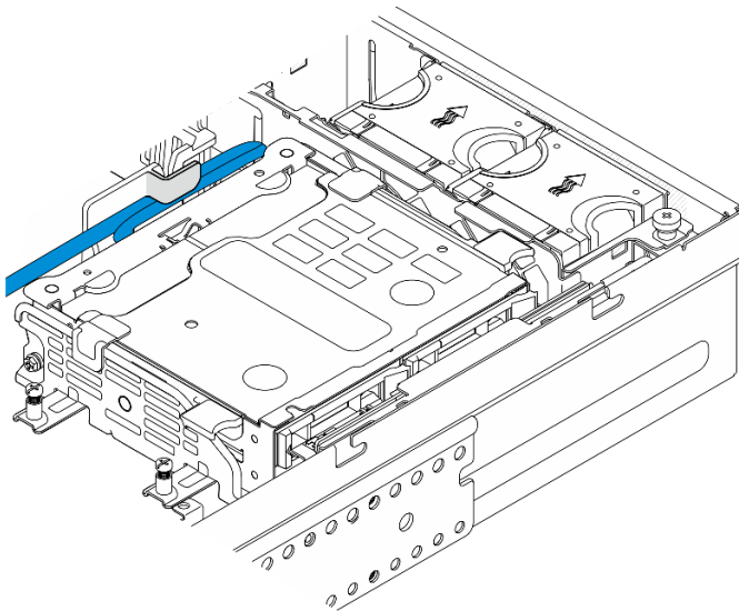
Abbildung 65. Mit der Kabelklemme der Prozessorluftführung gesicherte Kabel
