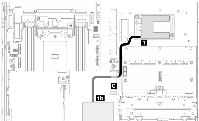
Abbildung 212. RAID-Adapter auf PCIe-Adapterkarte 2
