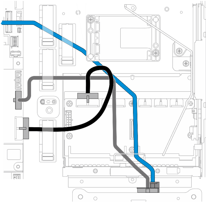
Abbildung 225. Kabelführung der vorderen Rückwandplatine für Laufwerke
