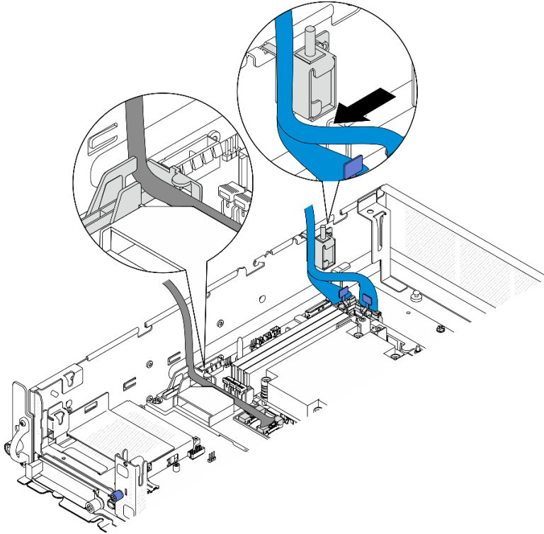
Abbildung 208. Kabelführung für PCIe-Adapterkarte 1
