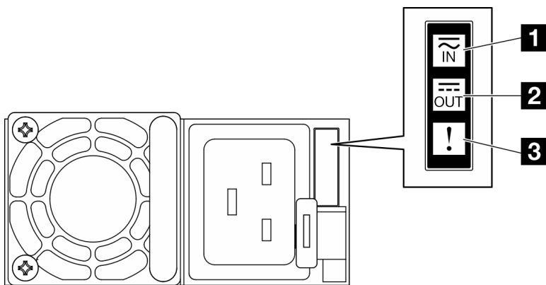
Abbildung 232. Netzteilanzeigen
