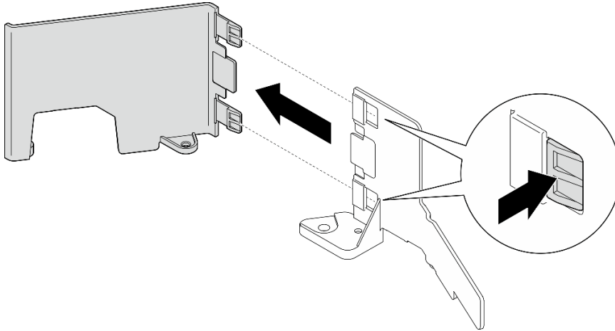
Abbildung 27. Teile der M.2-Luftführung trennen
