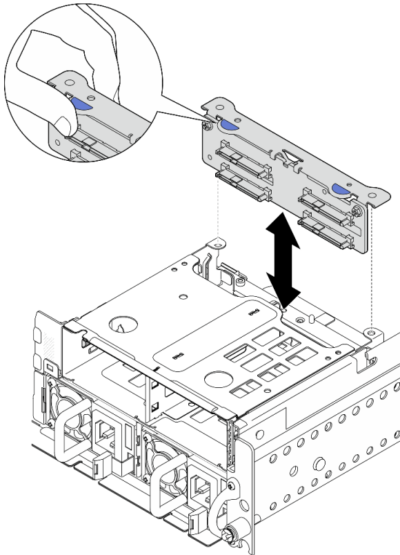
Abbildung 56. Vordere Rückwandplatine entfernen
