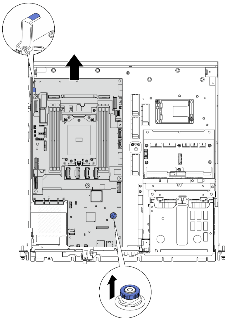
Figure 186. Retrait de la carte mère
