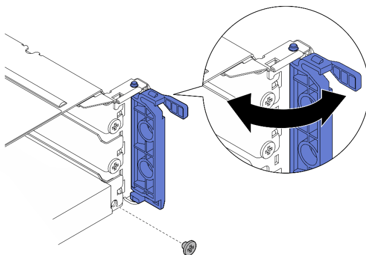
Figure 126. Installation des vis de fixation
