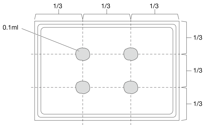
Figure 160. Application de la pâte thermoconductrice
