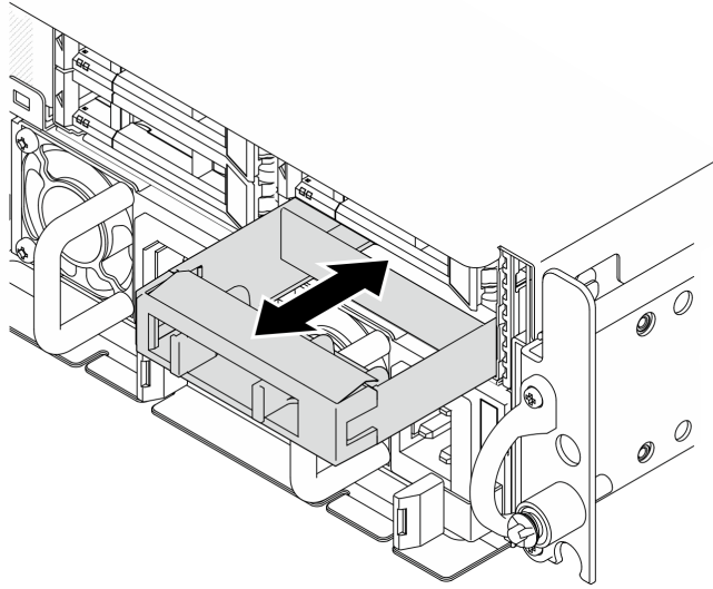
Figure 55. Installation d'un obturateur d'unité
