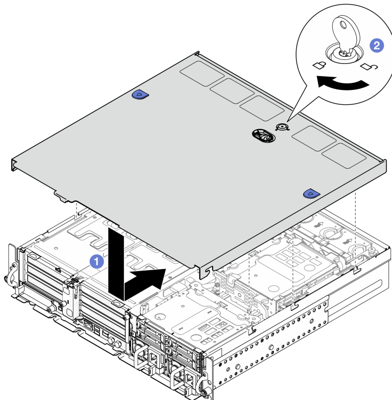
Figure 193. Installation du carter supérieur
