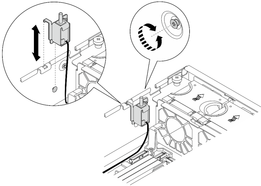
Figure 79. Retrait du commutateur de détection d'intrusion avec câble
