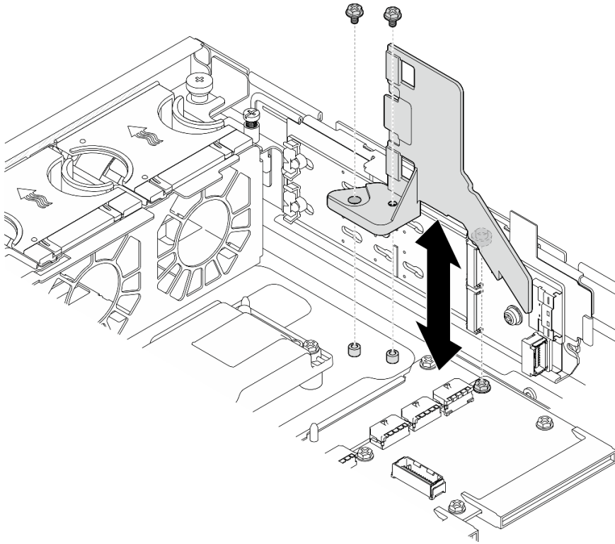
Figure 25. Retrait de la grille d'aération M.2 pour la configuration avec boîtier d'unités de disque dur interne
