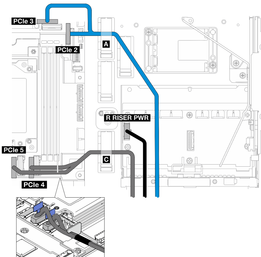
Figure 136. Cheminement des câbles du bloc mezzanine PCIe 2
