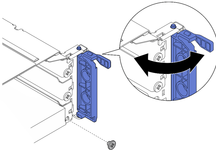
Figure 183. Installation des vis de fixation
