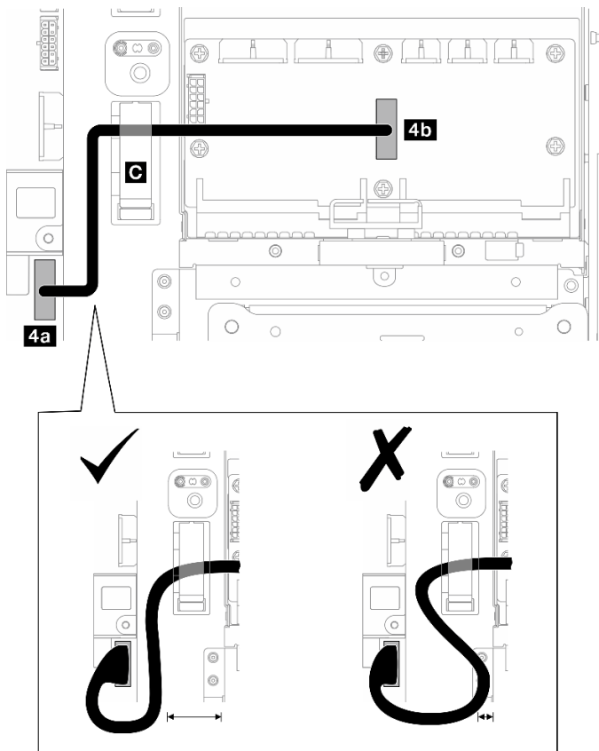
Figure 204. Cheminement des câbles de bande latérale PDB
