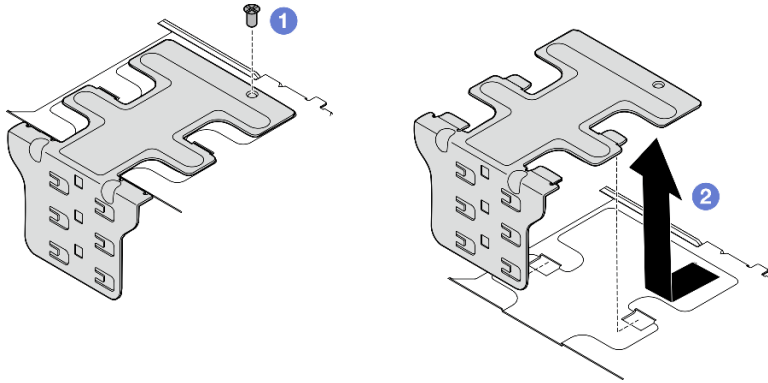
Figure 115. Retrait du support latéral
