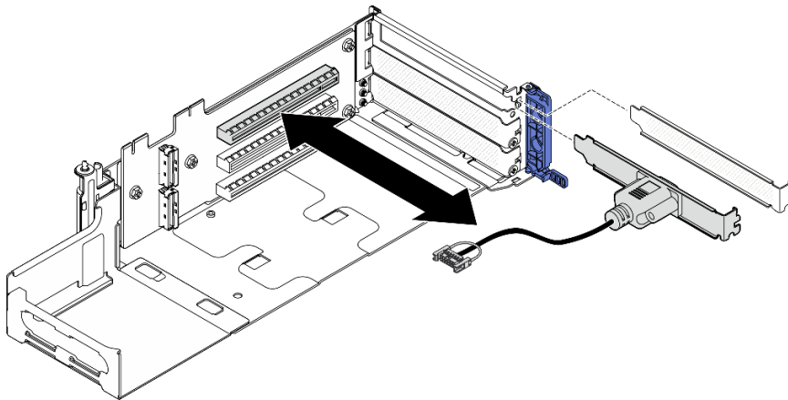
Figure 182. Installation du module de port série
