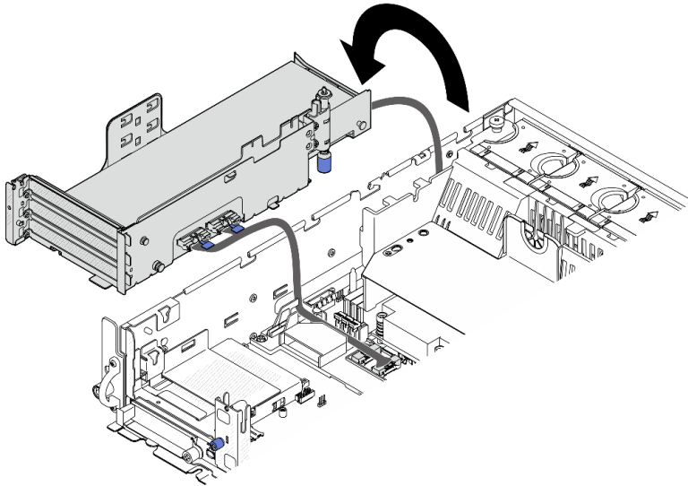
Figure 109. Placement de la carte mezzanine PCIe 1 à l'écart du châssis
