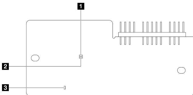
Figure 234. Voyants du module de microprogramme et de sécurité RoT
