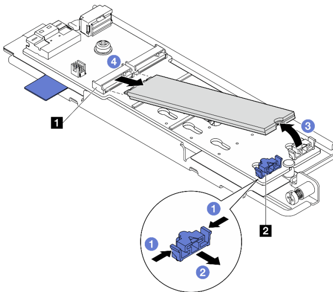
Figure 85. Retrait d'une unité M.2
