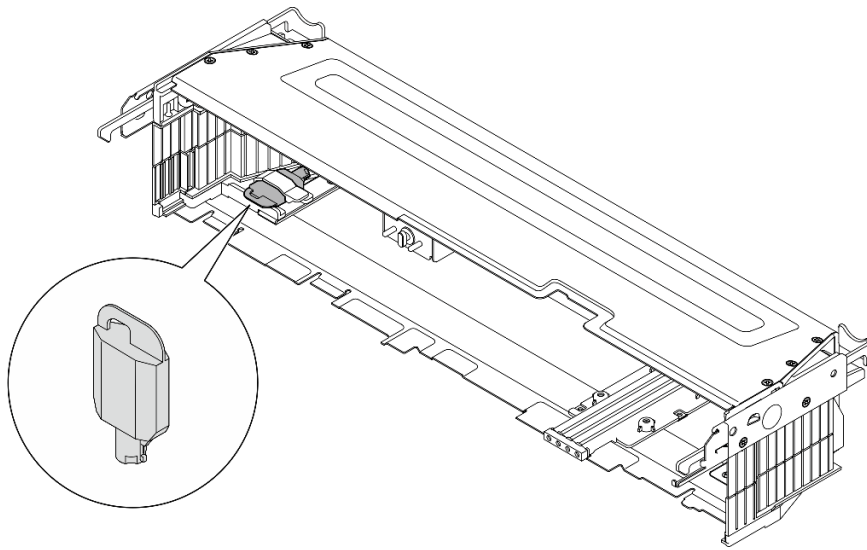
Figure 174. Emplacement de stockage de la clé du panneau de sécurité
