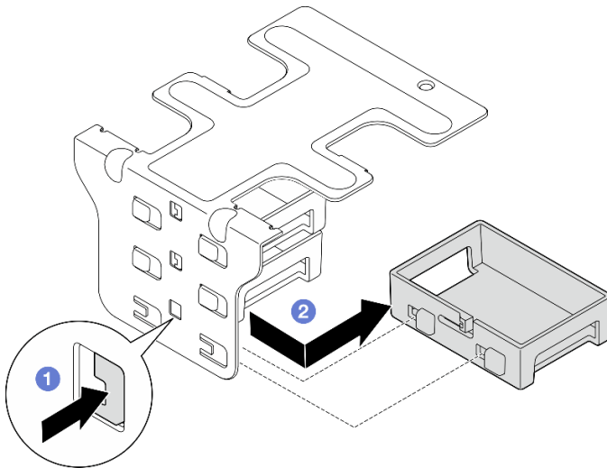
Figure 116. Retrait d'un obturateur extra-plat
