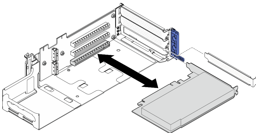
Figure 124. Installation d'un adaptateur PCIe dans la carte mezzanine PCIe 1
