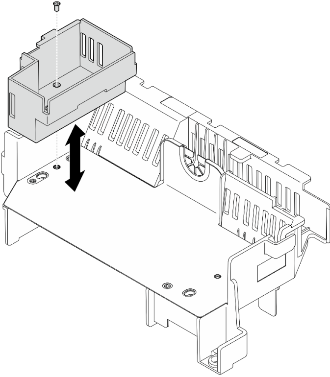
Figure 33. Remplacement de l'obturateur du de carte mezzanine 1
