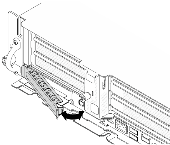
Figure 103. Installation de l'obturateur OCP
