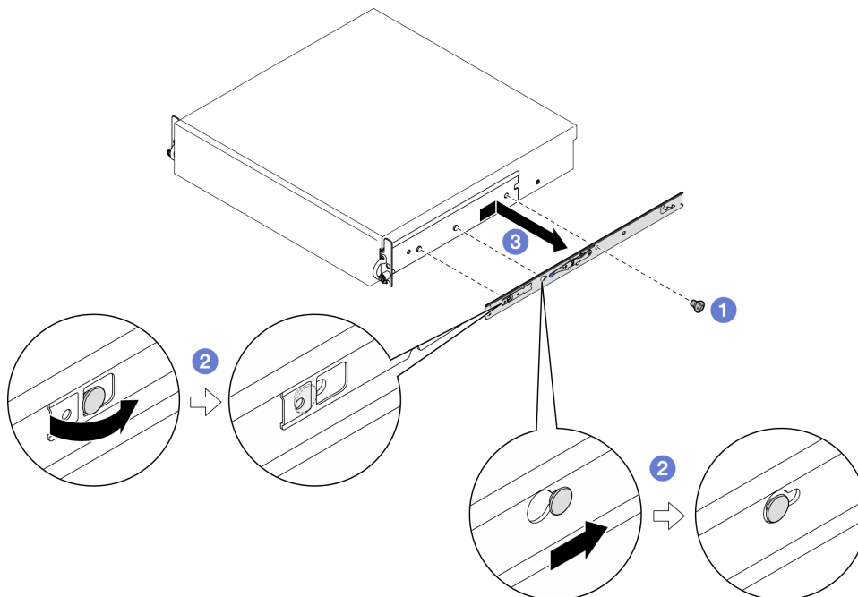
Figure 5. Retrait de la glissière interne
