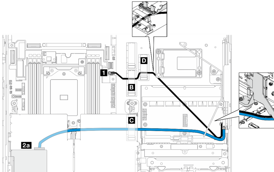
Figure 206. Adaptateur RAID sur la carte mezzanine PCIe 1
