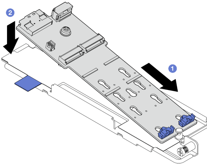
Figure 88. Installation du fond de panier M.2
