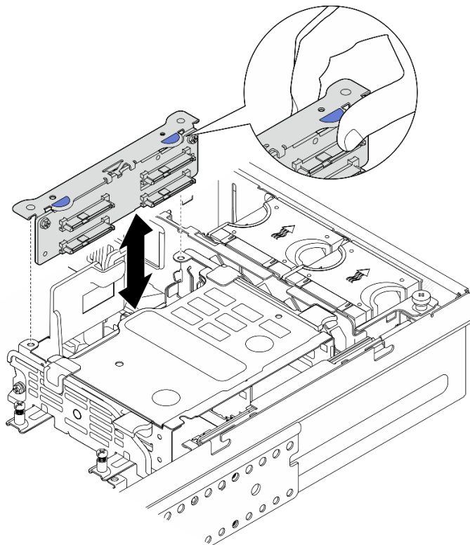
Figure 111. Retrait du fond de panier d'unité interne
