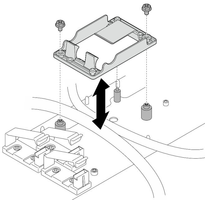
Figure 168. Retrait du support de module d'alimentation flash RAID
