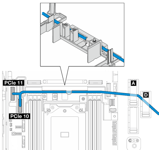
Figure 220. Câble de signal du fond de panier avant
