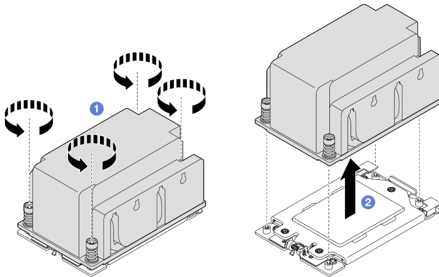
Figure 157. Retrait du dissipateur thermique 2U
