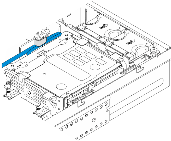
Figure 65. Câbles maintenus par le clip de fixation de la grille d'aération du processeur
