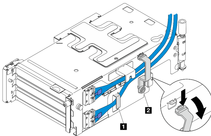
Figure 148. Cheminement des câbles du bloc mezzanine PCIe 2
