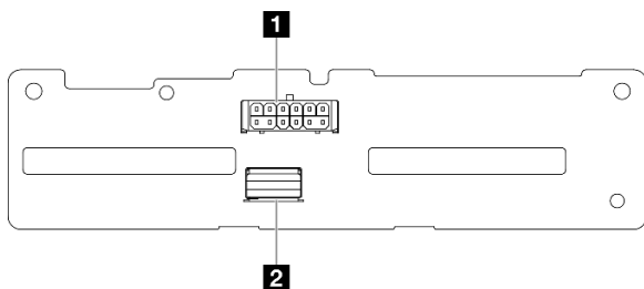
Figure 194. Connecteurs de fond de panier SAS/SATA
