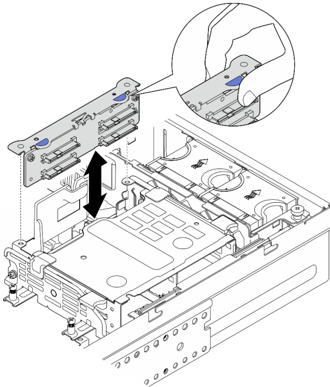
Figure 73. Installation du fond de panier d'unité interne
