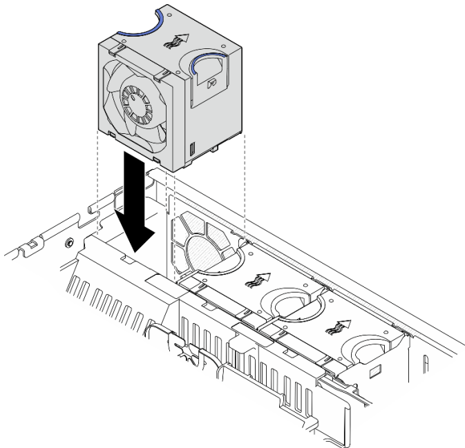
Figure 49. Installation d'un ventilateur
