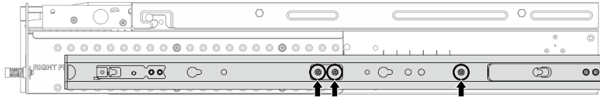
Figure 10. Trois vis pour la glissière interne de Kit de glissières ThinkEdge Friction 1 000 mm v2
