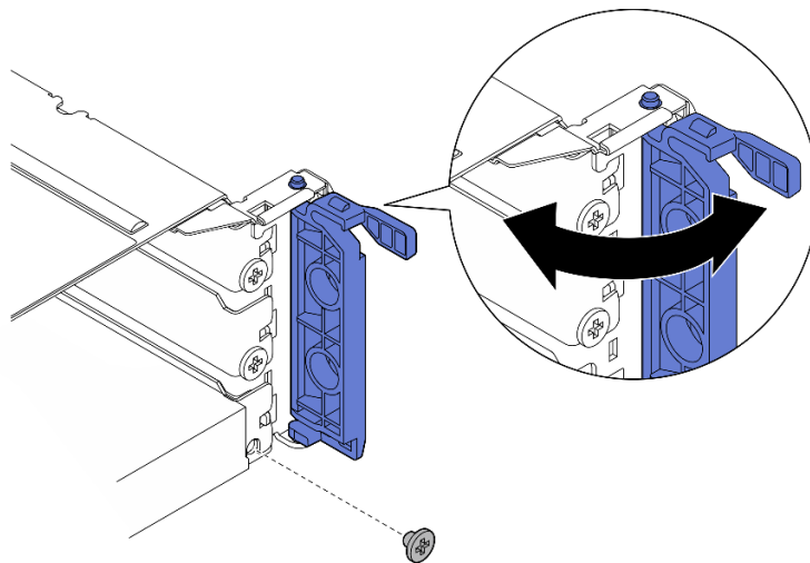
Figure 180. Retrait de la vis de retenue
