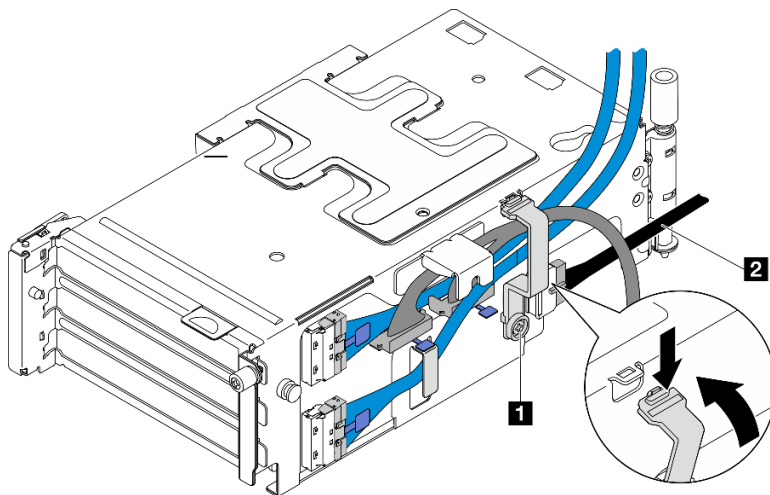
Figure 149. Cheminement des câbles du bloc mezzanine PCIe 2
