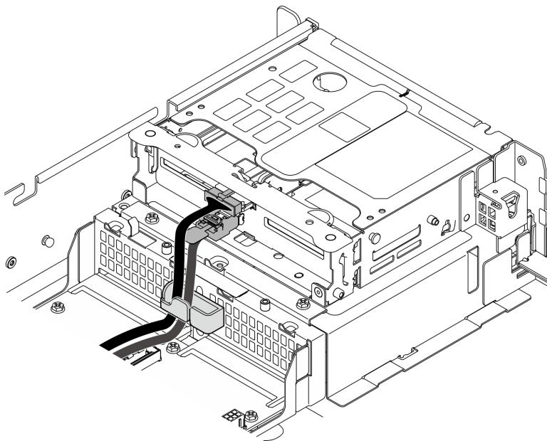
Figure 60. Cheminement des câbles du fond de panier d'unité avant
