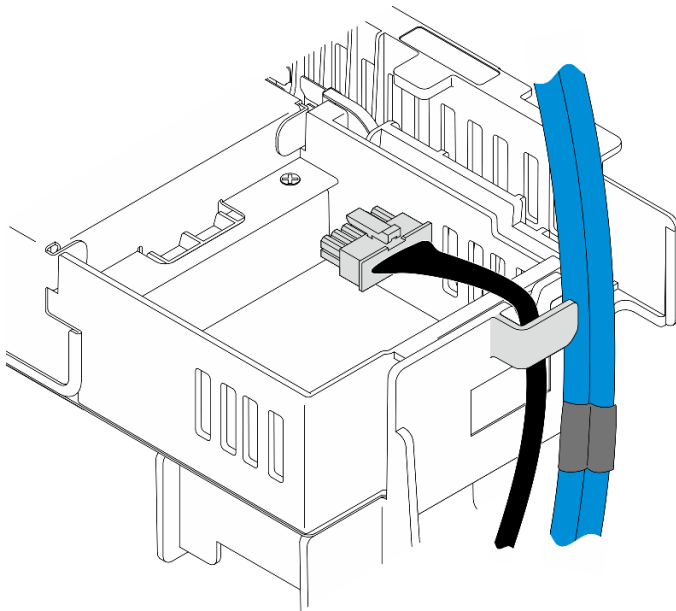
Figure 69. Câbles de fond de panier interne sur le clip de fixation
