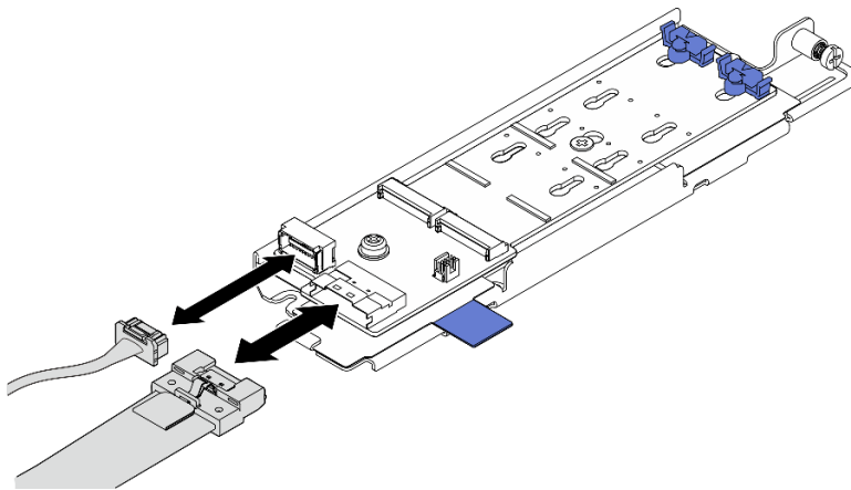
Figure 93. Connexion du câble au fond de panier M.2 SATA/x4 NVMe
