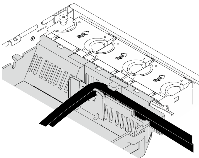
Figure 112. Cordons d'alimentation GPU sur la grille d'aération du processeur
