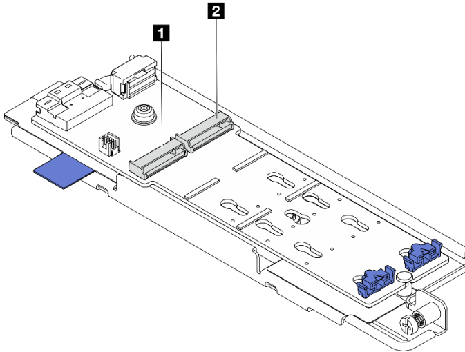
Figure 91. Numérotation des emplacements d'unités M.2
