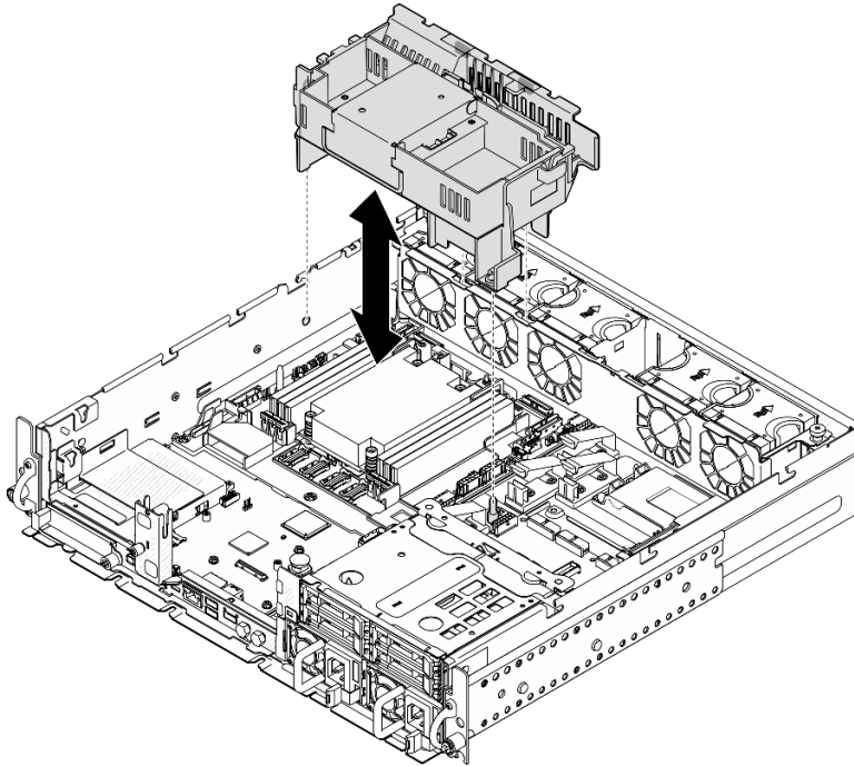
Figure 31. Retrait de la grille d'aération pour dissipateur thermique 1U
