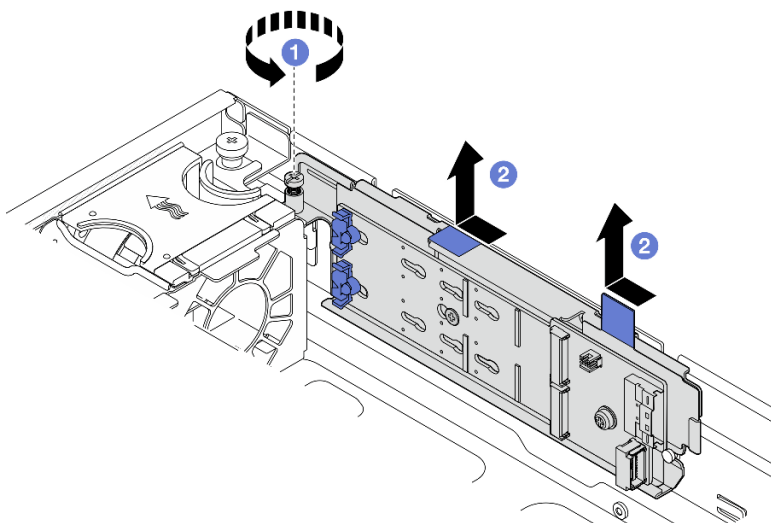
Figure 81. Retrait du fond de panier M.2
