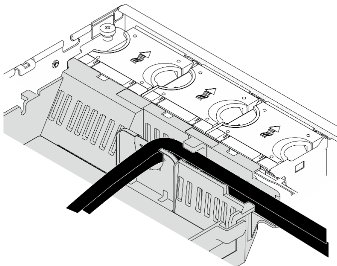
Figure 138. Cordons d'alimentation GPU sur la grille d'aération du processeur
