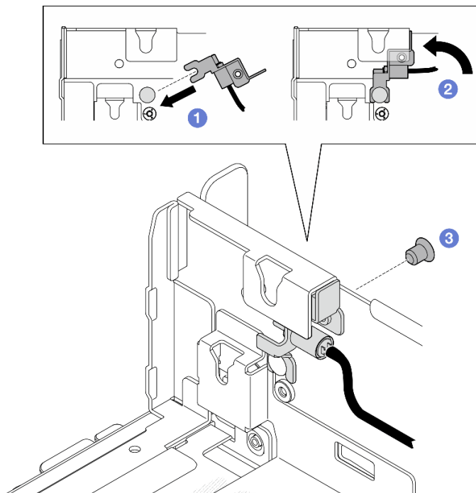
Figure 41. Installation du commutateur de détection de panneau
