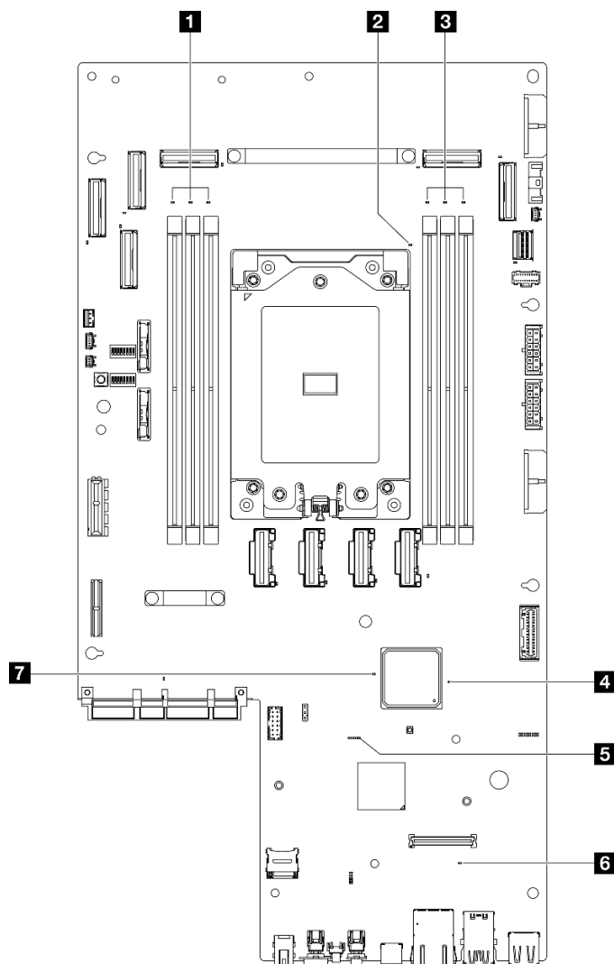
Figure 233. Voyants de la carte mère
