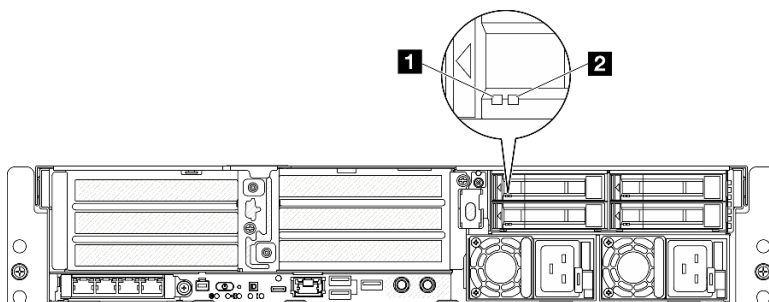
Figure 229. Voyants d'unité
