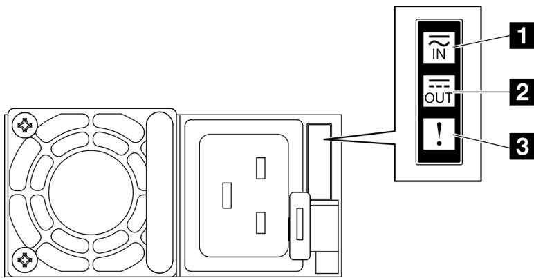
Figure 232. Voyants de l'alimentation
