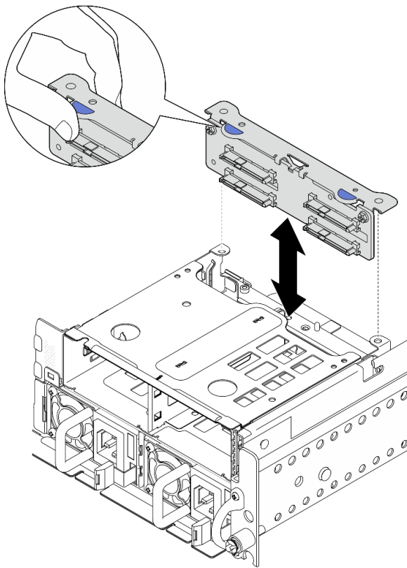
Figure 59. Installation du fond de panier d'unité avant
