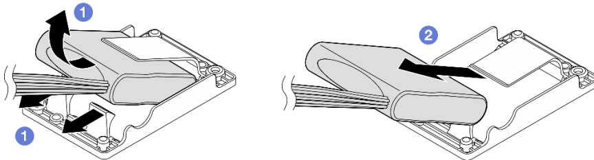
Figure 163. Retrait du module d'alimentation flash RAID
