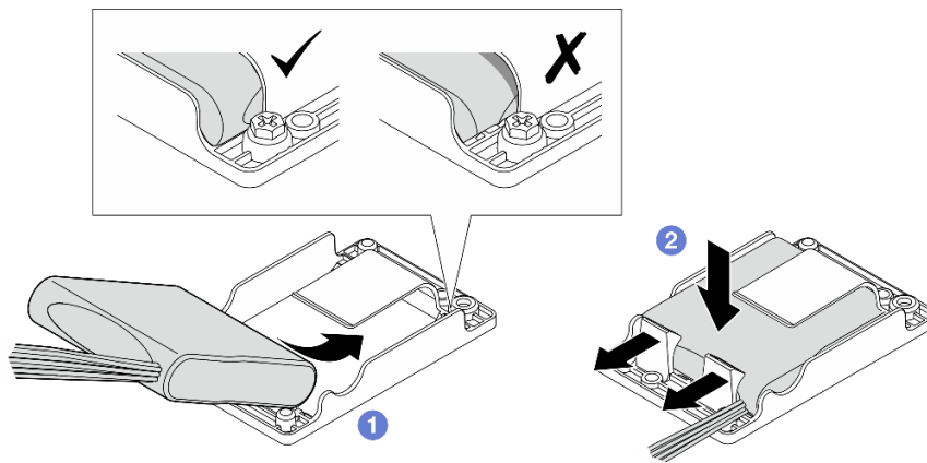
Figure 166. Installation du module d'alimentation flash RAID
