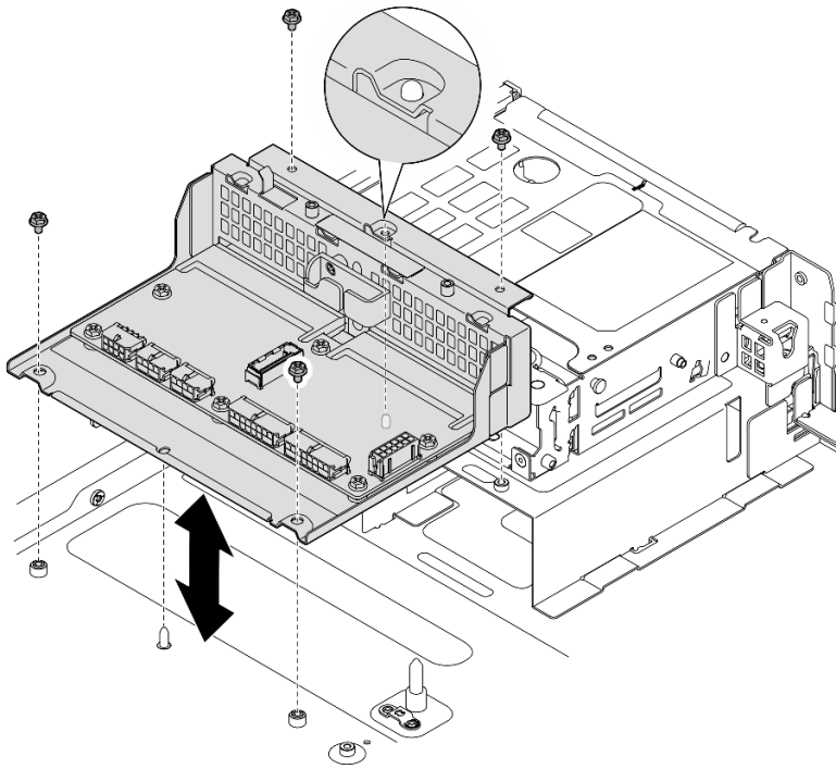
Figure 152. Installation du boîtier de PDB
