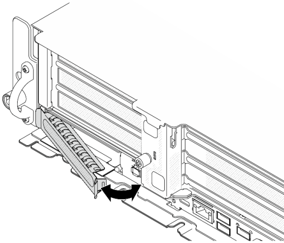
Figure 104. Retrait de l'obturateur OCP
