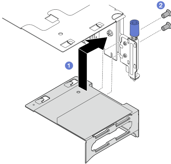
Figure 122. Installation de l'extension sur la carte mezzanine PCIe 1
