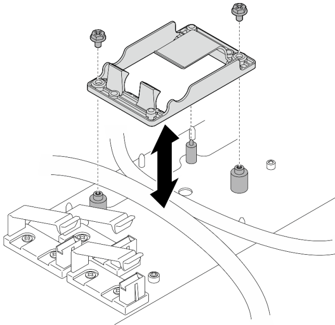
Figure 169. Installation du support de module d'alimentation flash RAID
