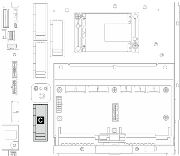
Figure 214. Clip de fixation C
