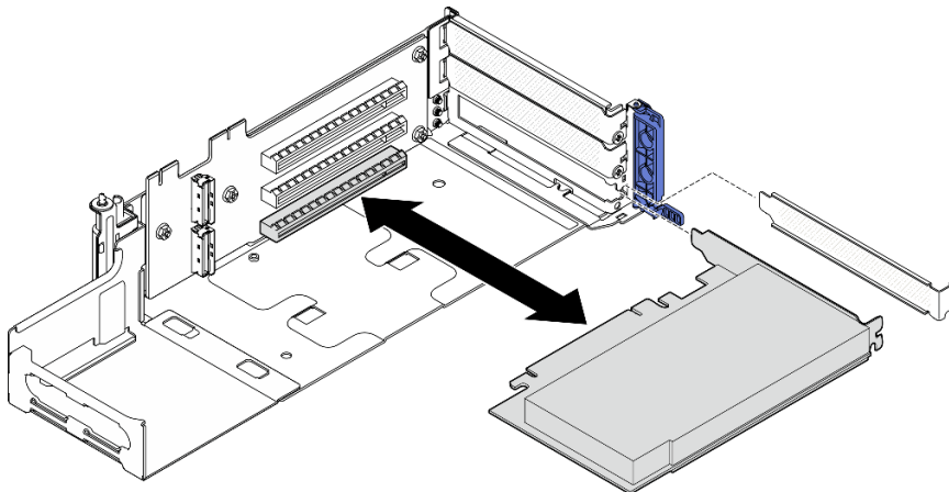
Figure 118. Retrait d'un adaptateur PCIe de la carte mezzanine PCIe 1
