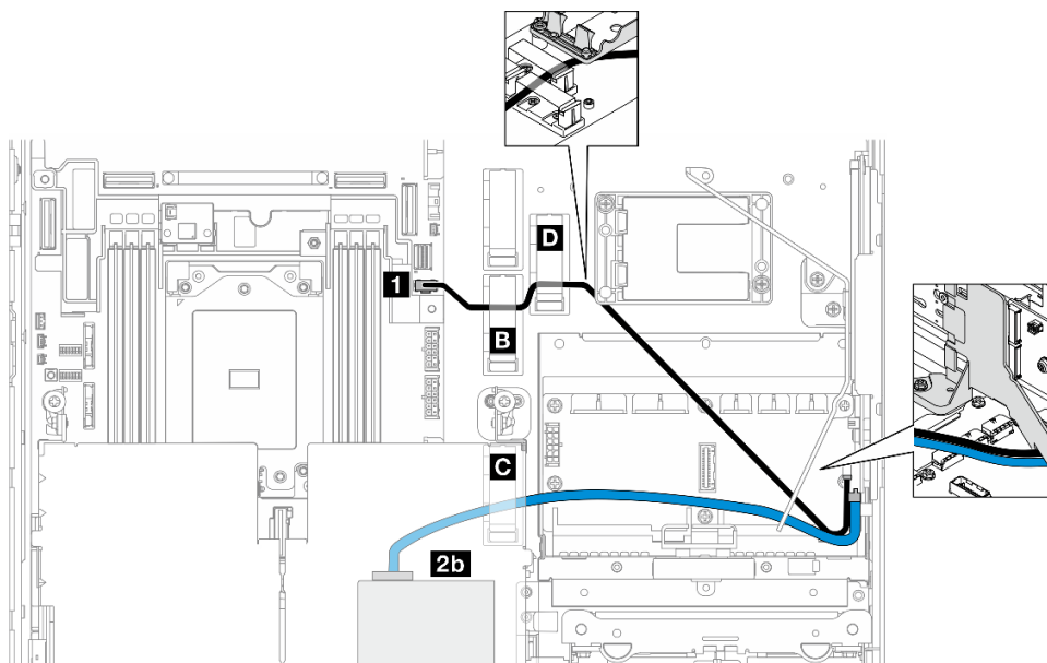
Figure 207. Adaptateur RAID sur la carte mezzanine PCIe 2
