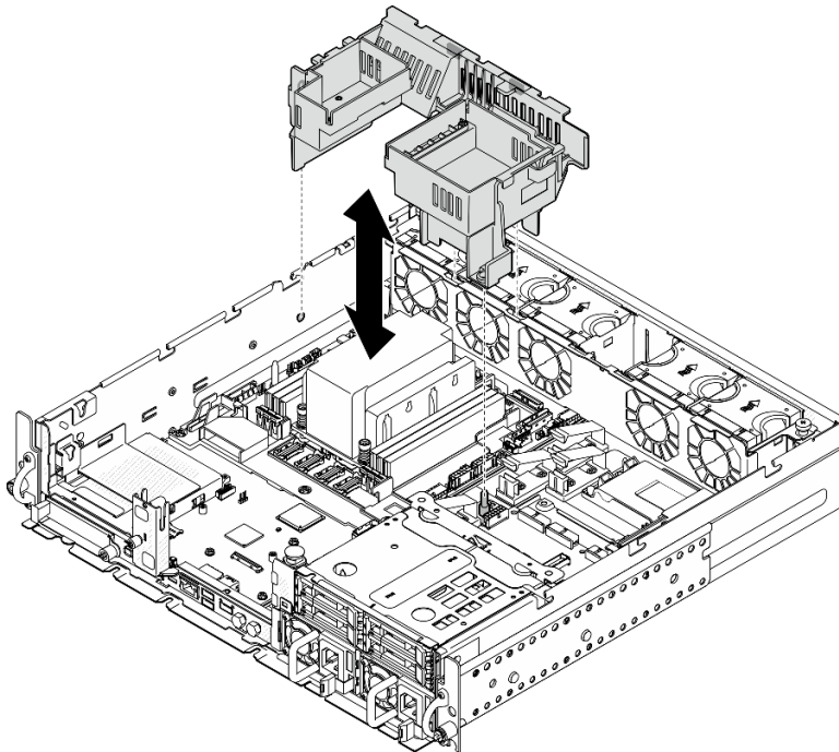
Figure 32. Retrait de la grille d'aération pour dissipateur thermique 2U
