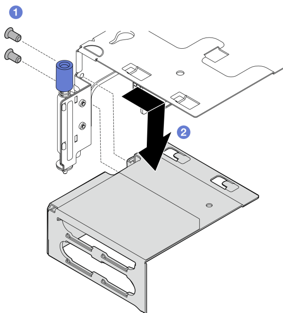
Figure 121. Retrait de l'extension de la carte mezzanine PCIe 2
