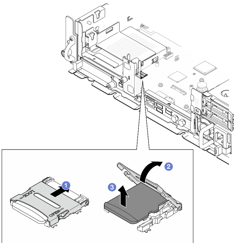
Figure 100. Retrait de la carte microSD
