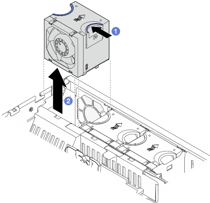
Figure 48. Retrait d'un module ventilateur
