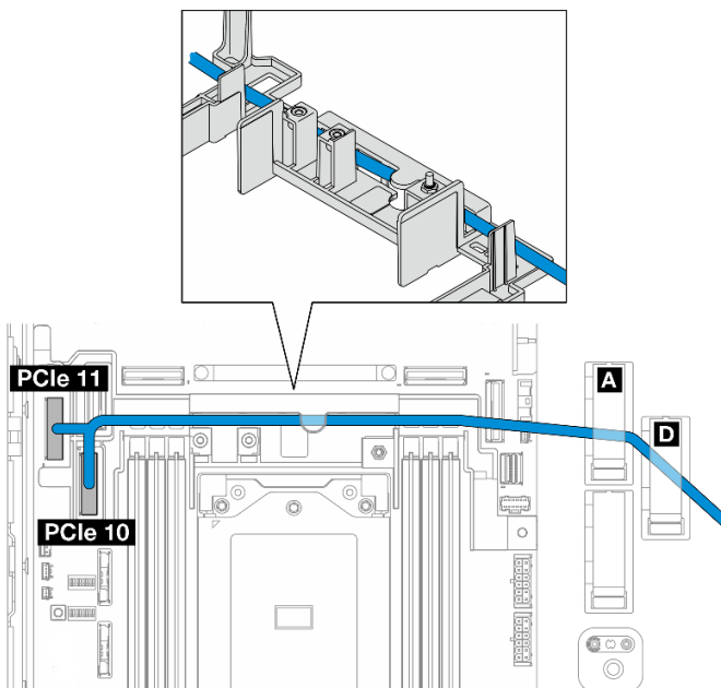
Figure 222. Câble de signal du fond de panier avant
