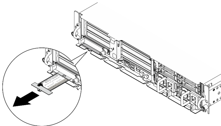
Figure 190. Étiquette d'accès réseau Lenovo XClarity Controller figurant sur l'étiquette amovible
