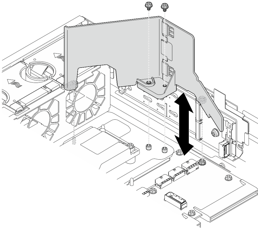
Figure 26. Retrait de la grille d'aération M.2 pour la configuration sans boîtier d'unités de disque dur interne
