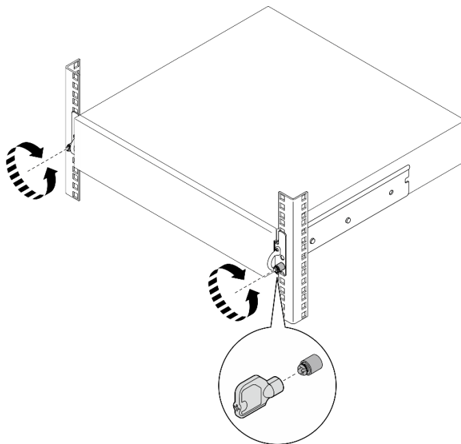
Figure 24. Fixation du serveur à l'armoire : supports EIA de sécurité
