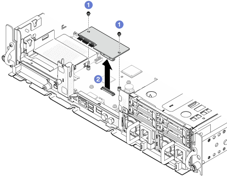
Figure 184. Retrait du module de microprogramme et de sécurité RoT
