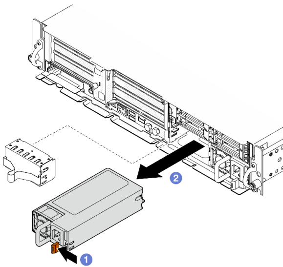
Figure 154. Retrait d'un bloc d'alimentation
