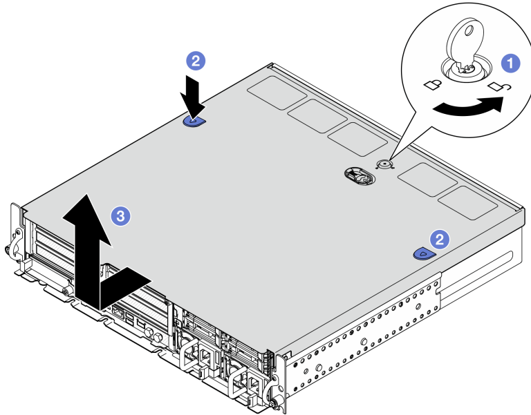
Figure 192. Retirer le carter supérieur
