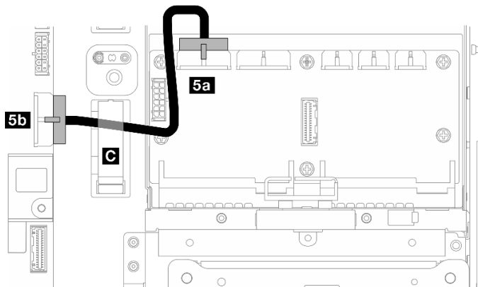
Figure 205. Cheminement des câbles de la carte mère 1
