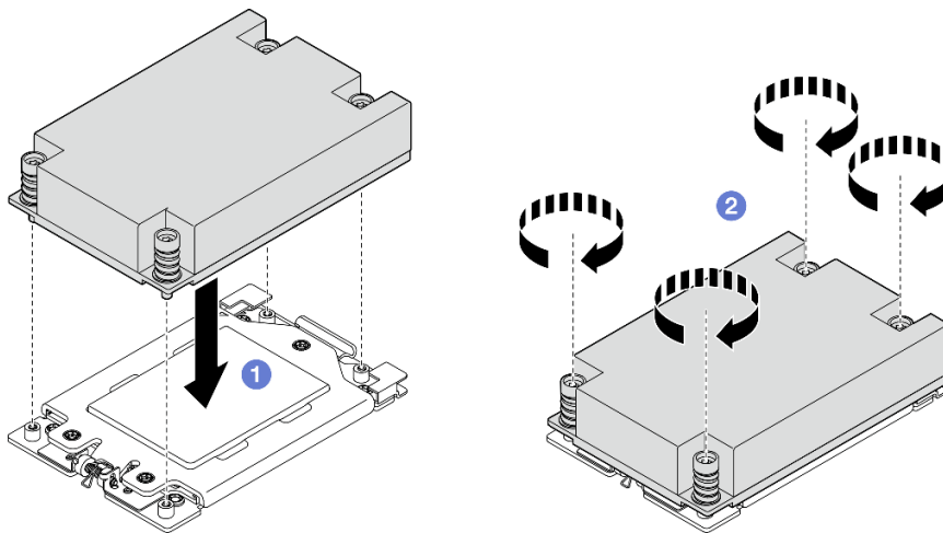
Figure 161. Installation du dissipateur thermique 1U
