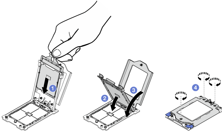
Figure 159. Installation d'un processeur
