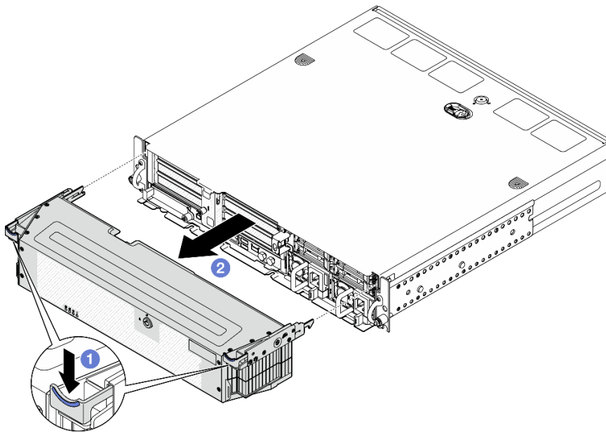
Figure 171. Retrait du panneau de sécurité
