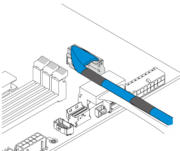
Figure 219. Câble de signal du fond de panier interne
