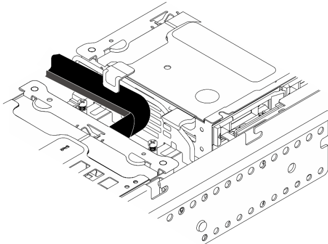
Figure 75. Cheminement des câbles du fond de panier d'unité avant
