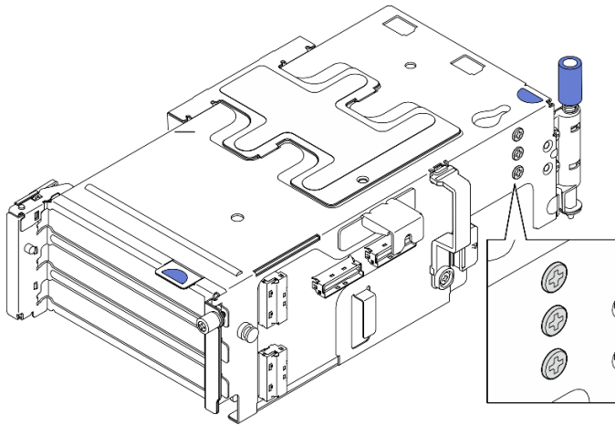
Figure 128. Vis de rechange sur carte mezzanine PCIe 2
