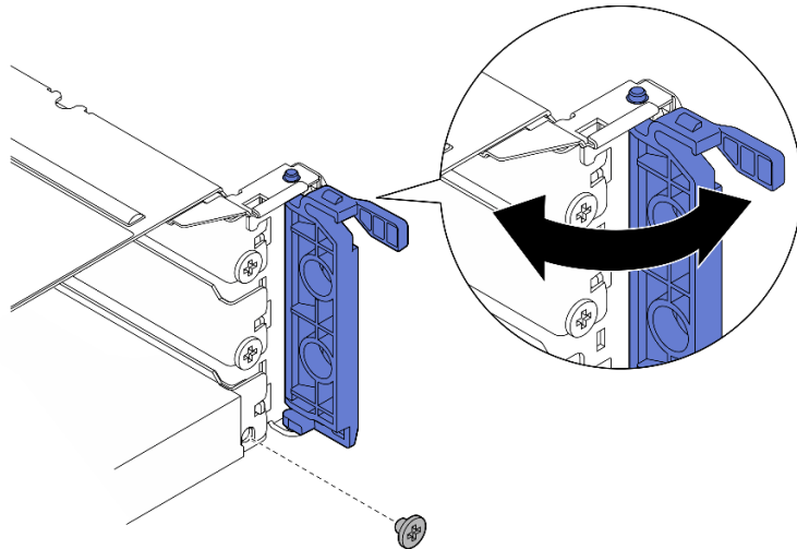
Figure 117. Retrait de la vis de retenue
