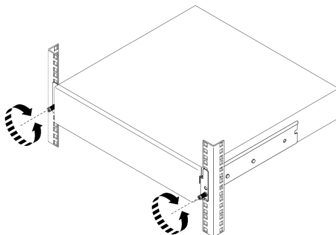
Figure 23. Fixation du serveur à l'armoire : supports EIA standards
