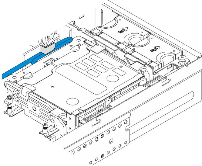
Figure 74. Cheminement des câbles du fond de panier d'unité interne
