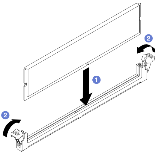
Figure 99. Installation d'un module de mémoire
