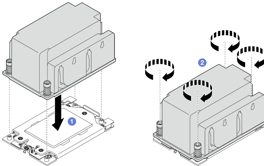
Figure 162. Installation du dissipateur thermique 2U
