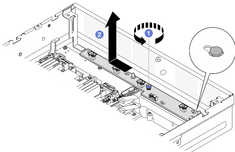
Figure 51. Retrait de la carte de contrôleur de ventilation
