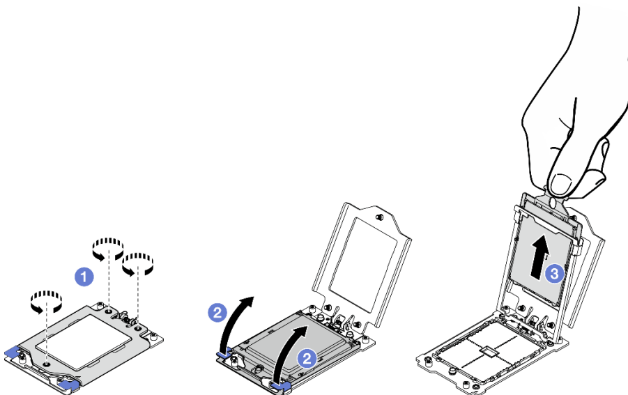
Figure 158. Retrait d'un processeur
