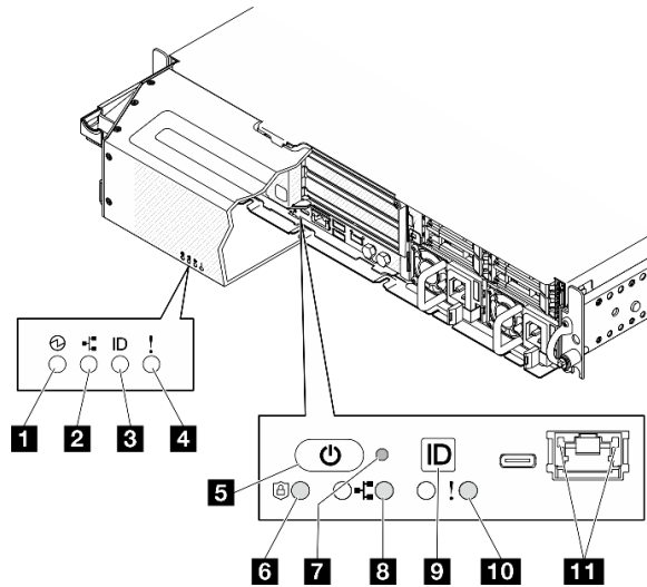
Figure 230. Voyants avant
