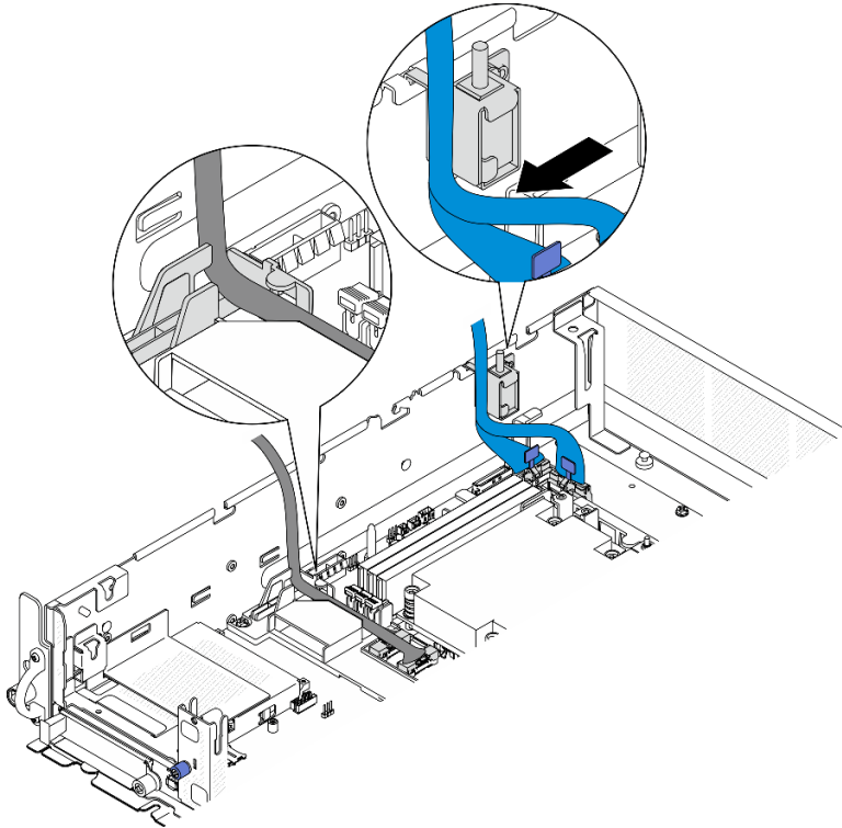
Figure 208. Cheminement des câbles du bloc mezzanine PCIe 1
