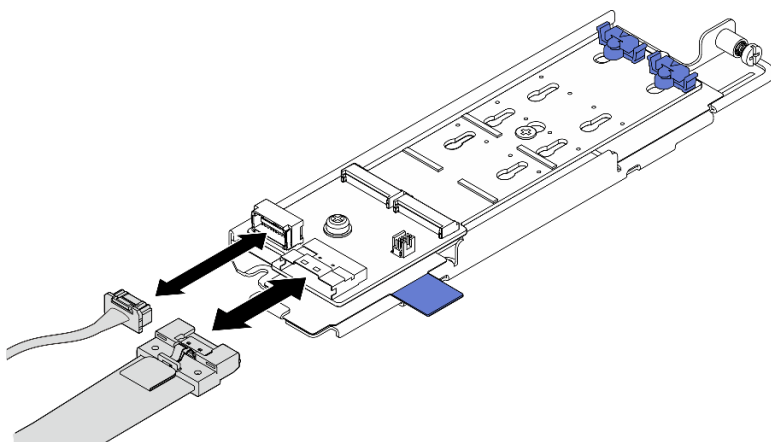
Figure 82. Déconnexion du câble du fond de panier M.2 SATA/x4 NVMe
