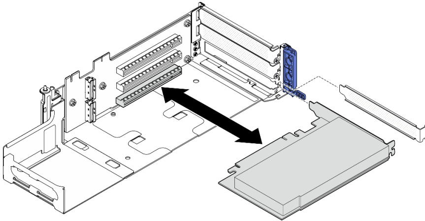
图 118. 从 PCIe 转接卡 1 上卸下 PCIe 适配器
