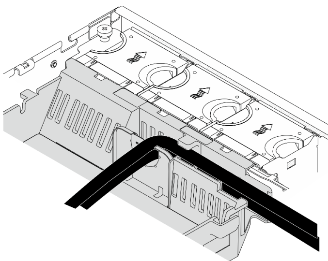
图 138. 处理器导风罩上的 GPU 电源线
