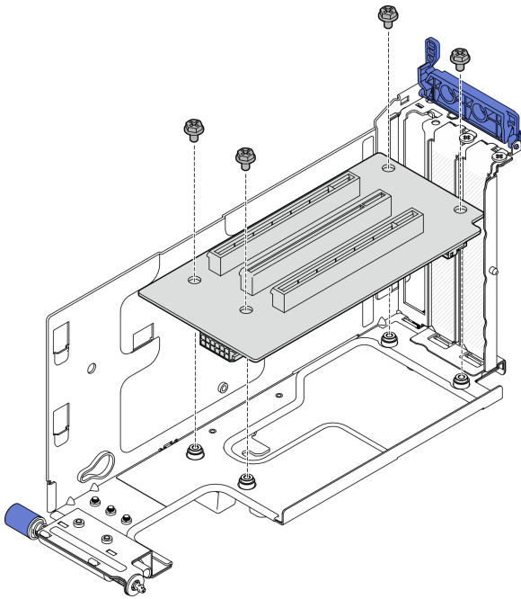
图 143. 从 PCIe 转接卡 2 上卸下转接卡
