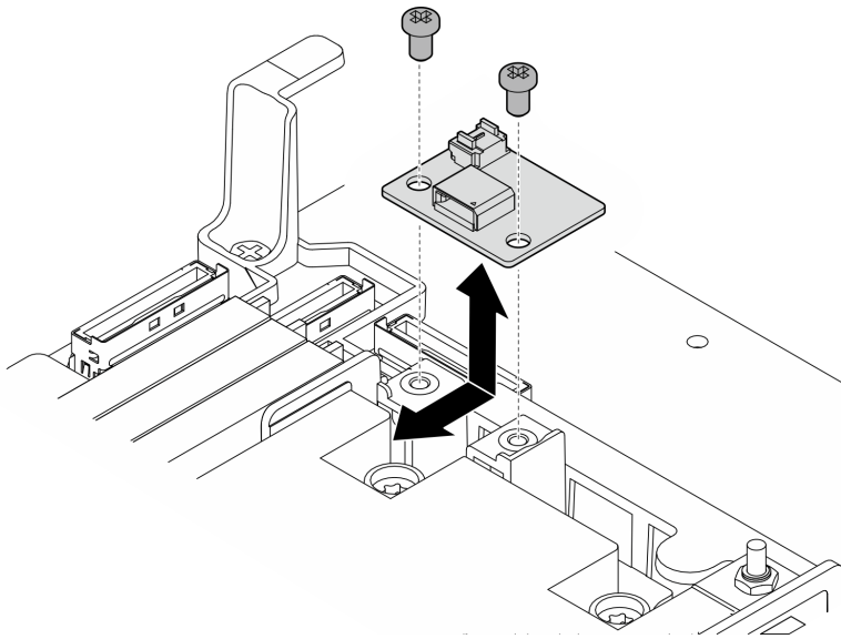
图 38. 卸下气流传感器板
