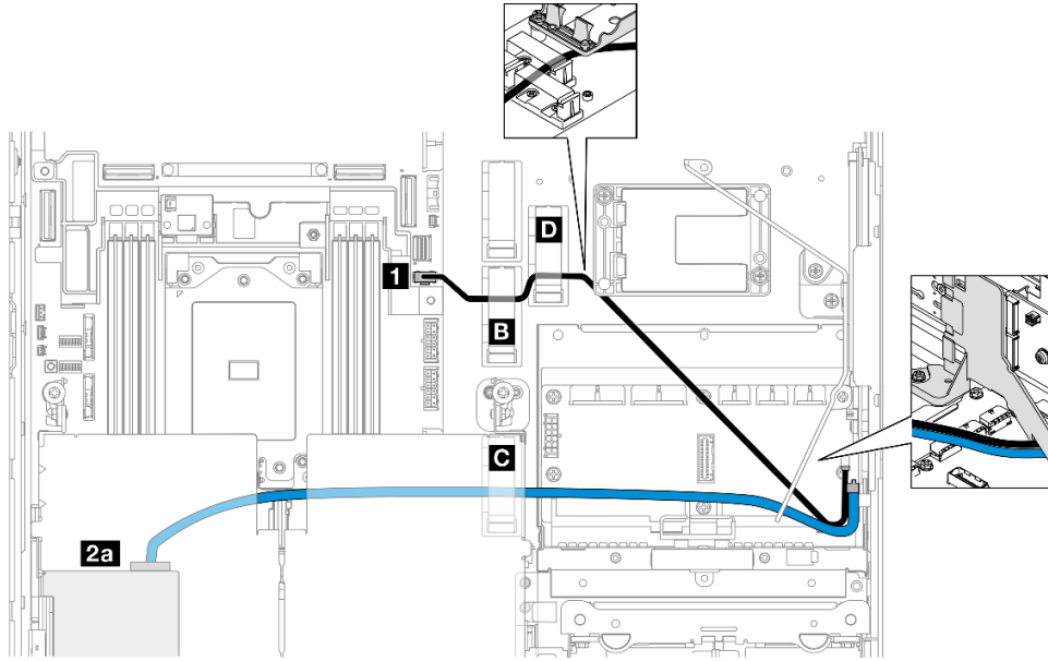
图 206. PCIe 转接卡 1 上的 RAID 适配器
