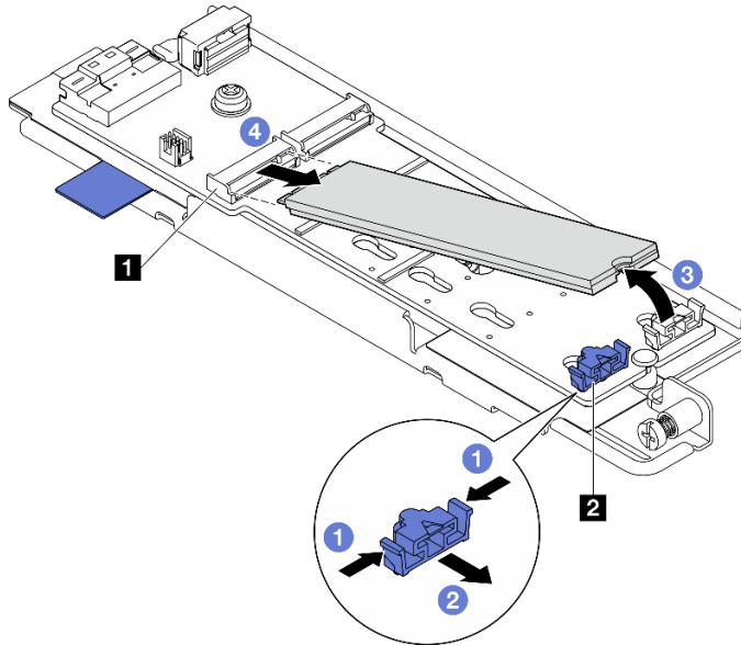
图 85. 卸下 M.2 硬盘
