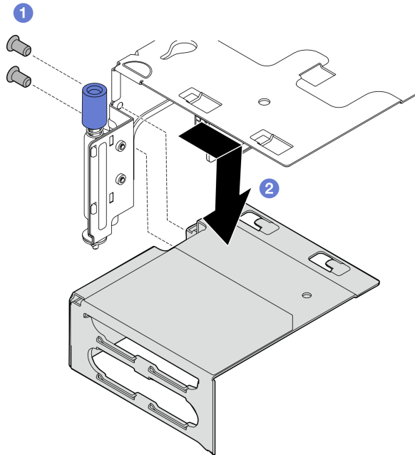
图 121. 从 PCIe 转接卡 2 上卸下扩展器
