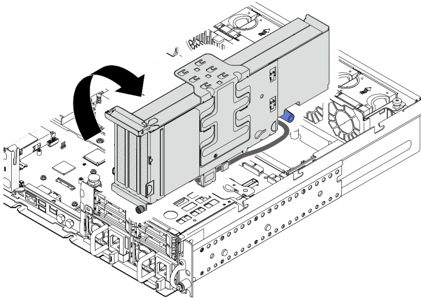
图 114. 将 PCIe 转接卡 2 放在机箱旁边
