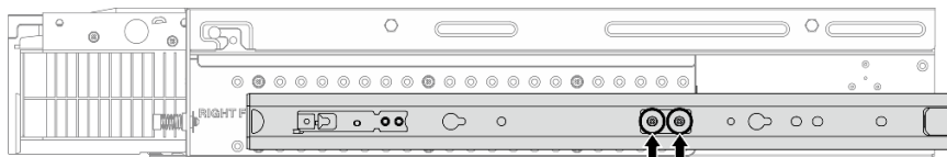
图 20. ThinkEdge 1000 毫米摩擦导轨套件 v2 的 inner 导轨有两颗螺钉
