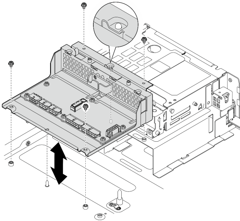
图 151. 卸下 PDB 架
