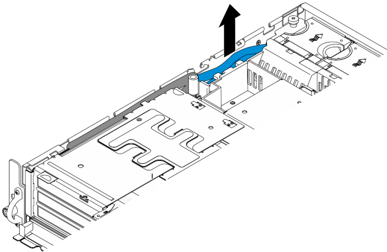
图 107. 取出 PCIe 转接卡 1 信号线缆
