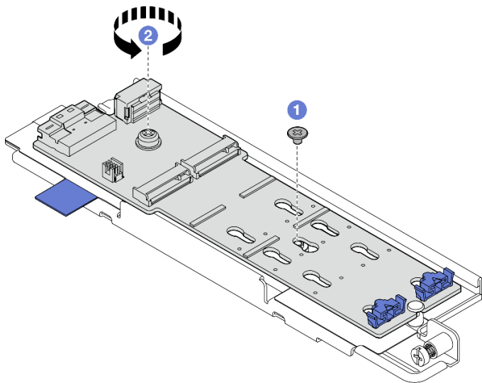
图 86. 卸下 M.2 背板
