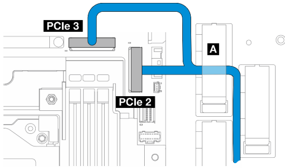
图 215. 内置背板信号线缆
