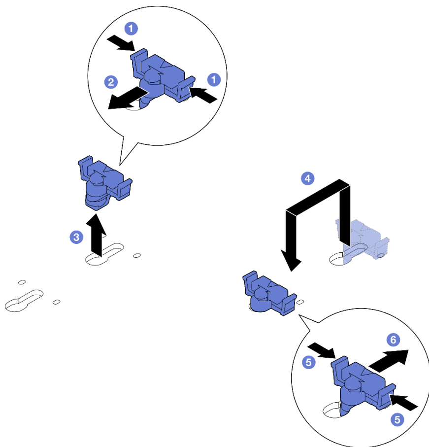
图 90. 调整 M.2 固定器
