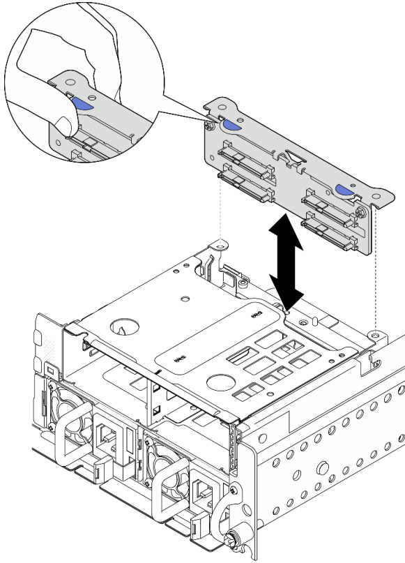
图 59. 安装正面硬盘背板
