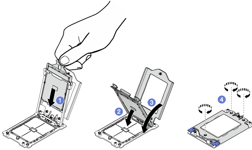
图 159. 安装处理器
