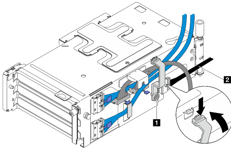
图 149. PCIe 转接卡 2 线缆布放
