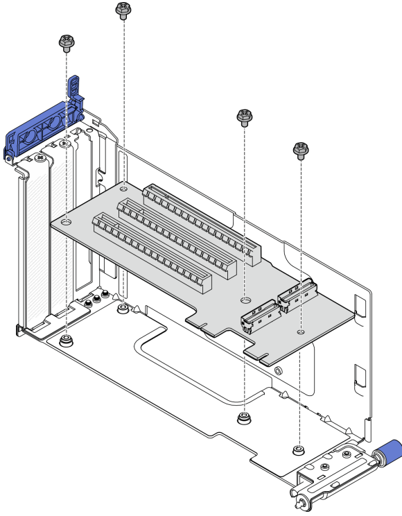
图 142. 从 PCIe 转接卡 1 上卸下转接卡
