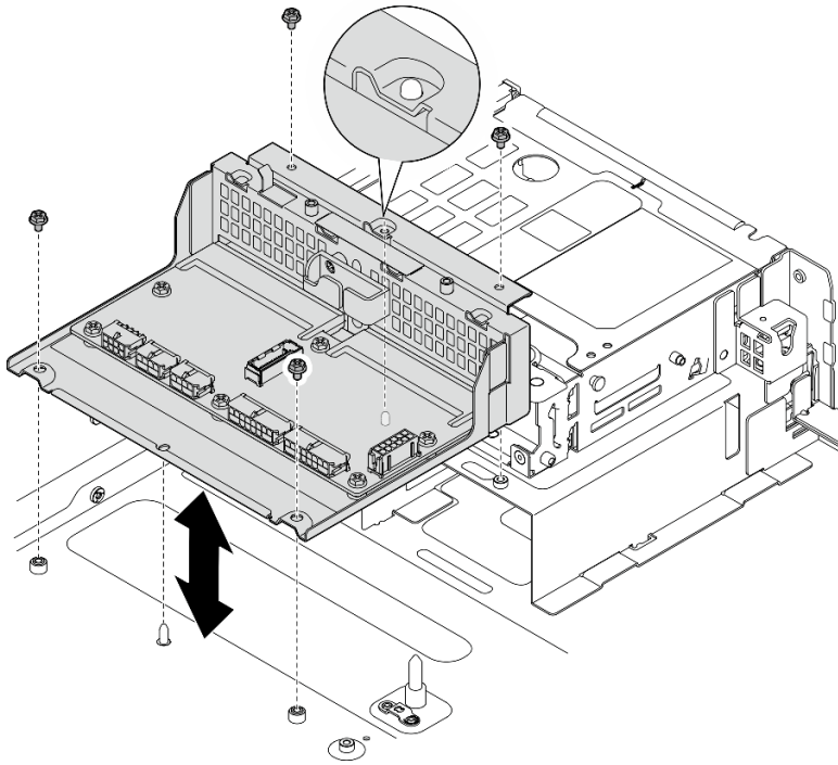
图 152. 安装 PDB 架
