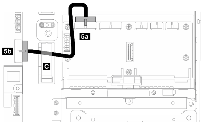
图 205. 主板电源 1 线缆布放
