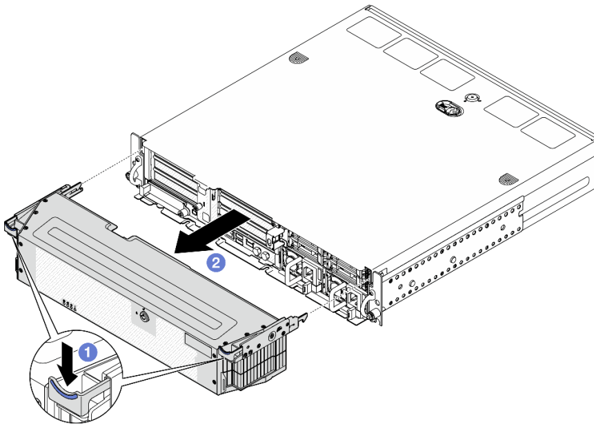
图 171. 卸下安全挡板
