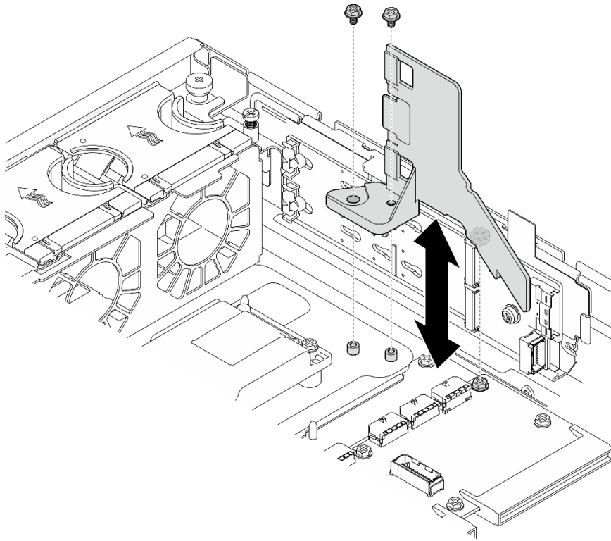
图 25. 为带有内置硬盘仓的配置卸下 M.2 导风罩
