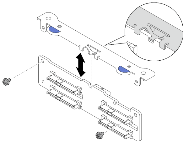
图 57. 从背板支架上拆下硬盘背板
