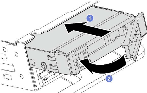
图 77. 安装内置硬盘
