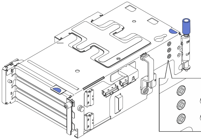
图 128. PCIe 转接卡 2 上的备用螺钉
