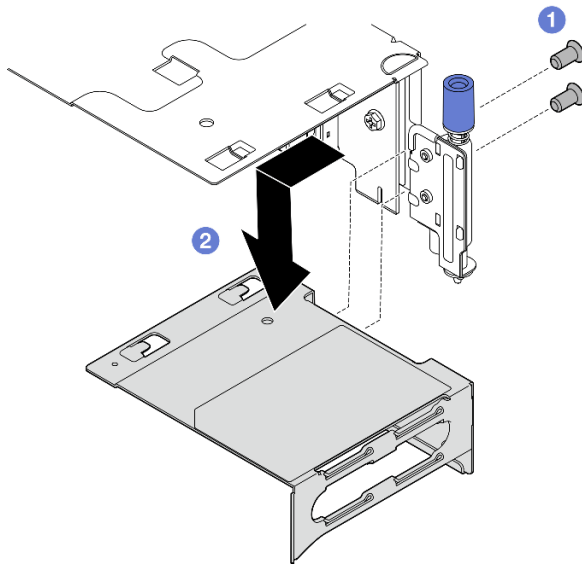
图 120. 从 PCIe 转接卡 1 上卸下扩展器
