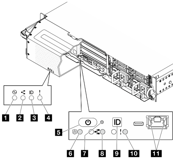
图 230. 正面 LED
