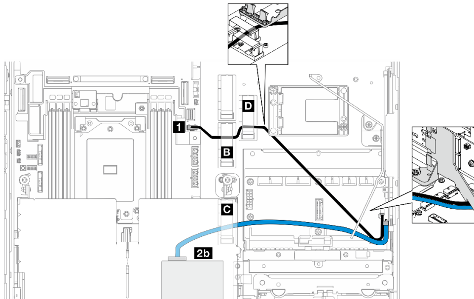
图 207. PCIe 转接卡 2 上的 RAID 适配器
