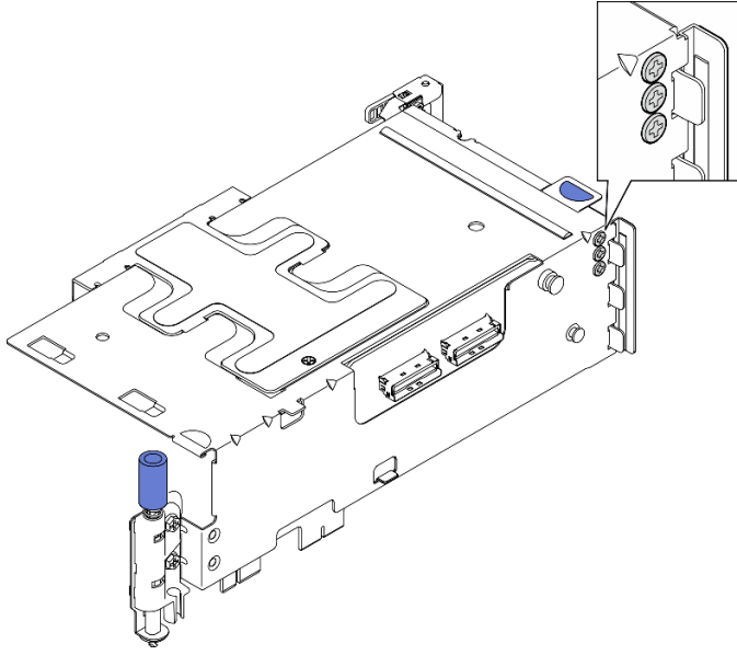
图 127. PCIe 转接卡 1 上的备用螺钉
