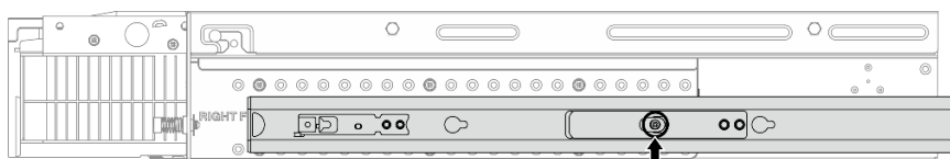
图 19. ThinkEdge 双柱摩擦导轨套件的 inner 导轨有一颗螺钉
