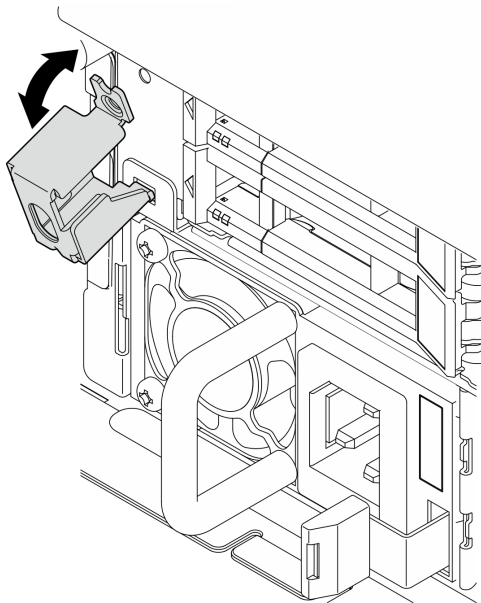
图 178. 安装安全挡板钥匙锁支架
