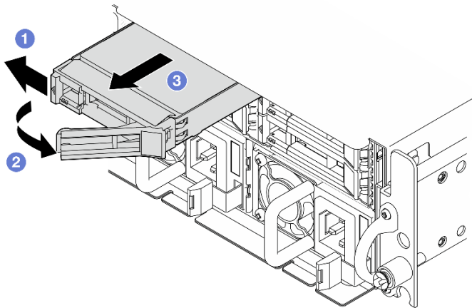
图 54. 卸下正面热插拔硬盘
