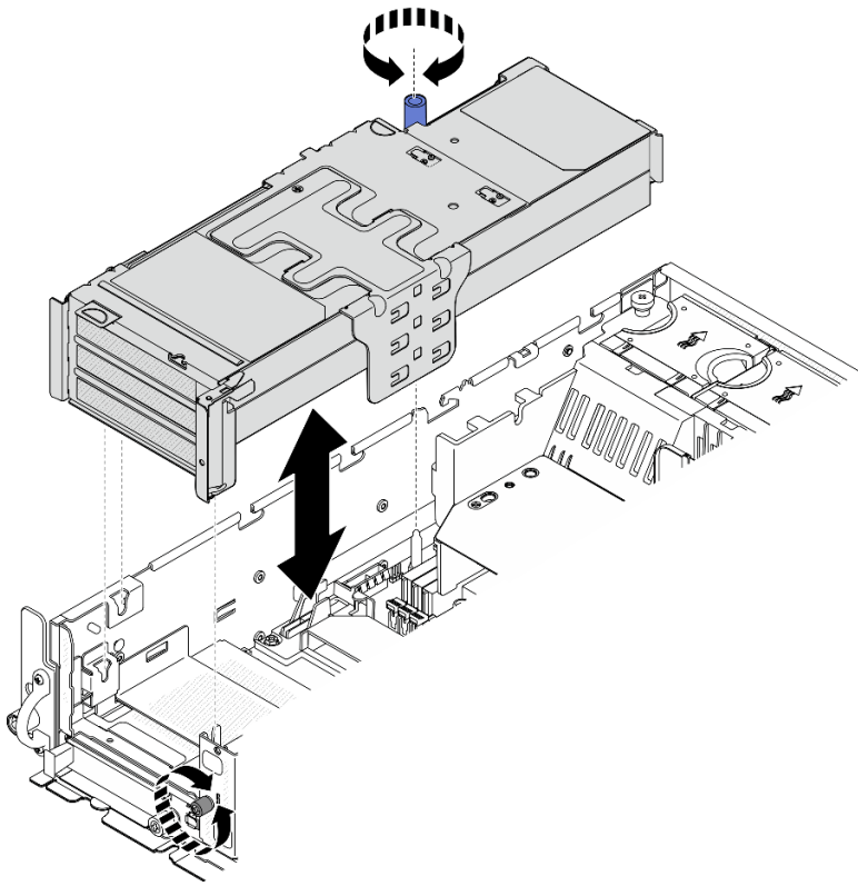
图 132. 安装 PCIe 转接卡 1
