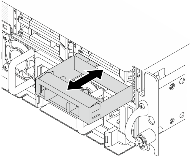
图 55. 安装硬盘填充件
