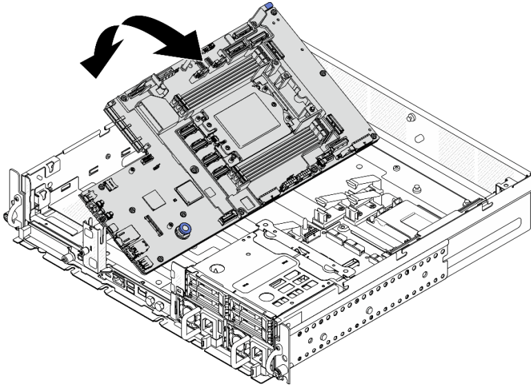
图 187. 卸下主板
