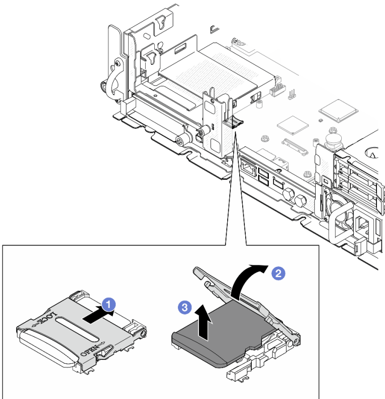
图 100. 卸下 MicroSD 卡
