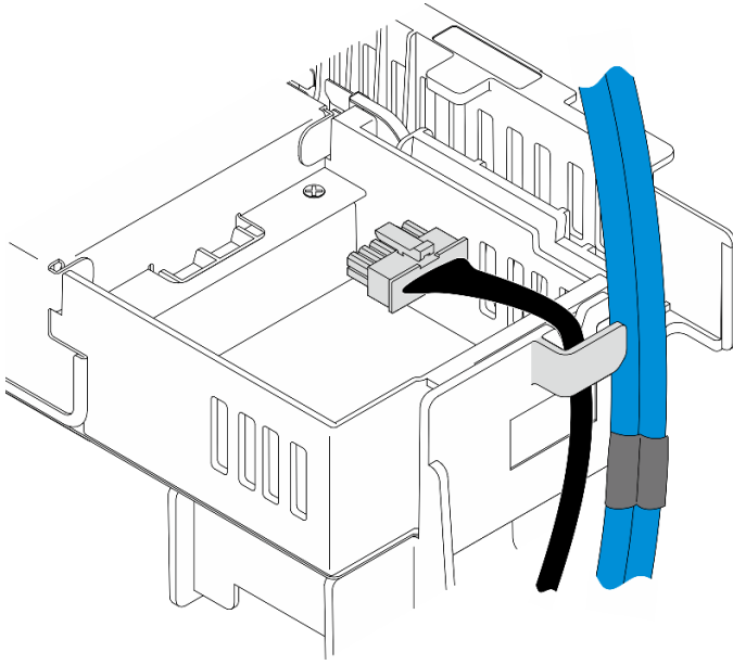
图 72. 线缆夹中的内置背板线缆
