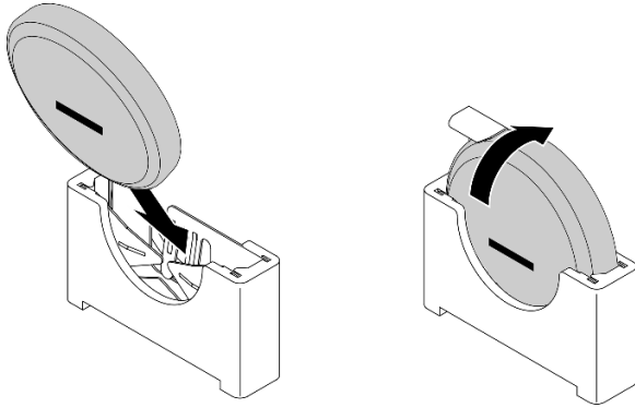
图 47. 安装 CMOS 电池
