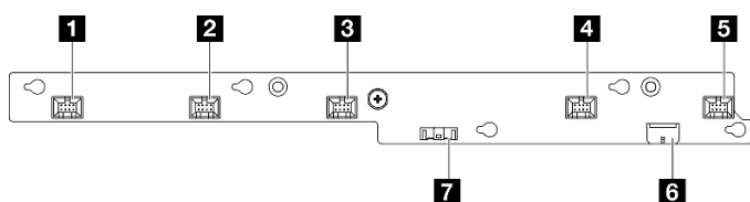
图 196. 风扇控制板接口
