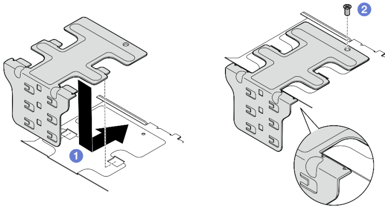
图 130. 安装侧面支架
