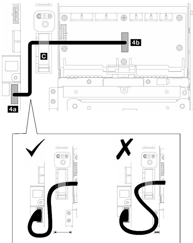
图 204. PDB 边带线缆布放
