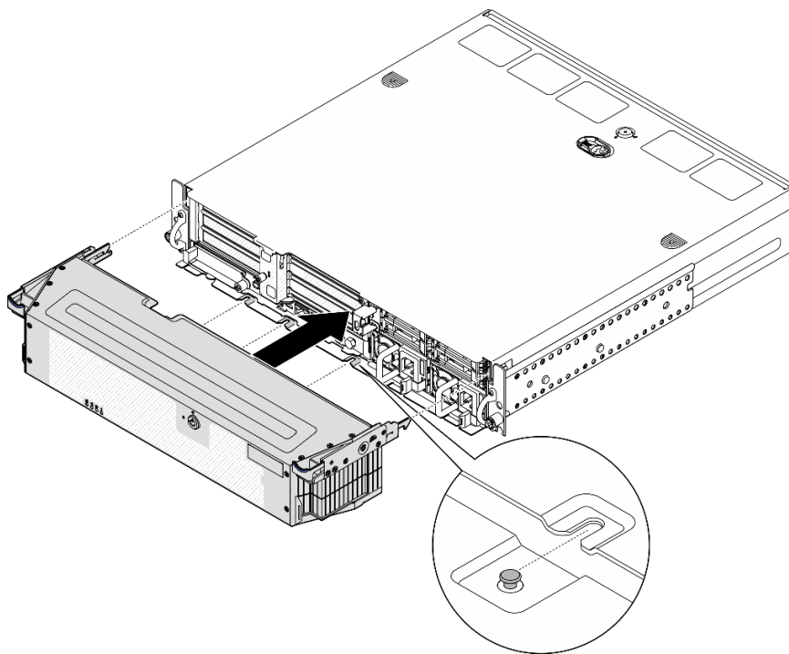
图 175. 安装安全挡板
