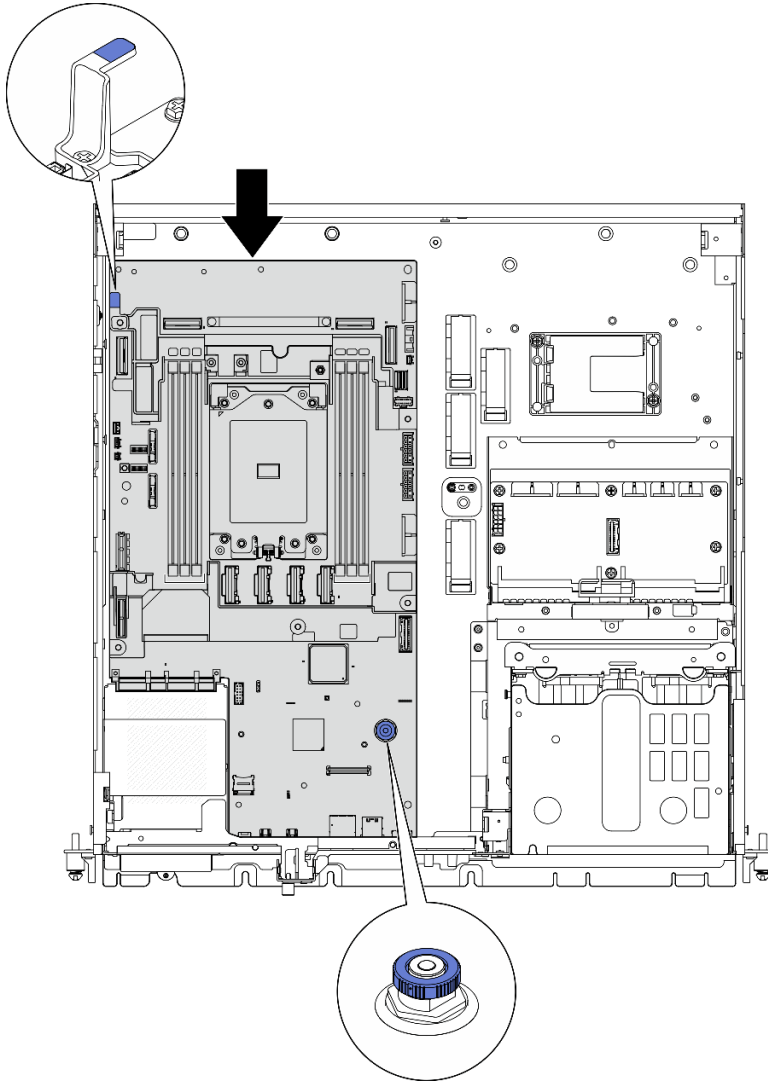
图 189. 固定主板
