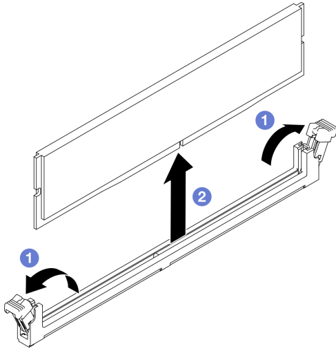
图 97. 卸下内存条
