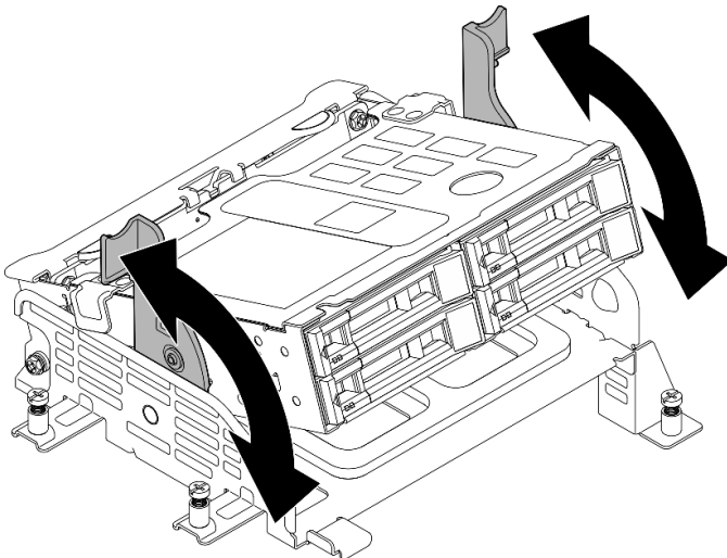
图 63. 转动内置硬盘仓
