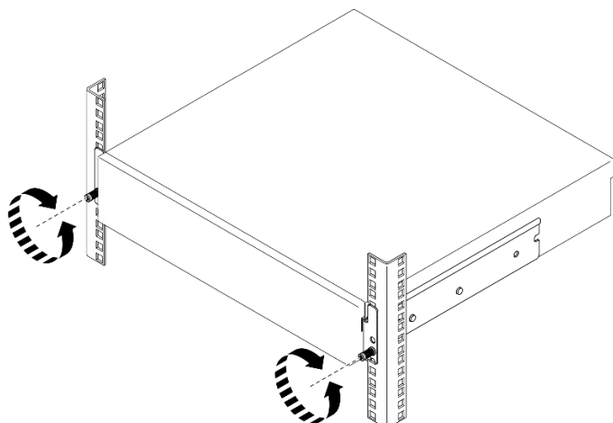
图 23. 将服务器固定到机架：标准 EIA 支架
