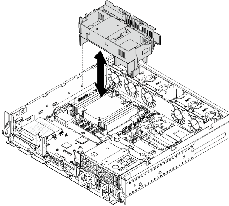
图 36. 为 1U 散热器安装导风罩
