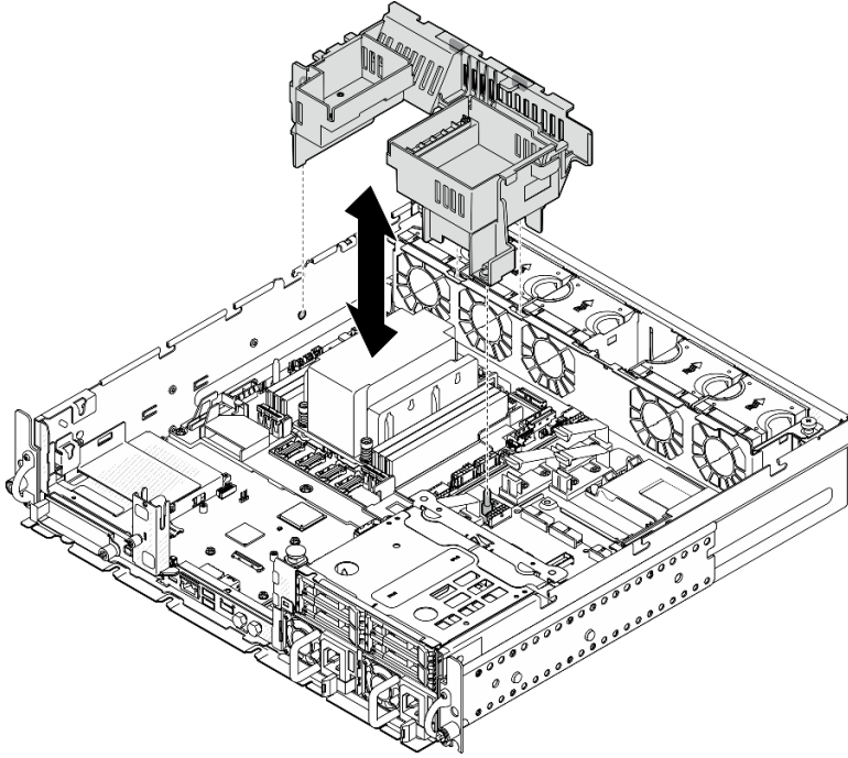
图 32. 为 2U 散热器卸下导风罩
