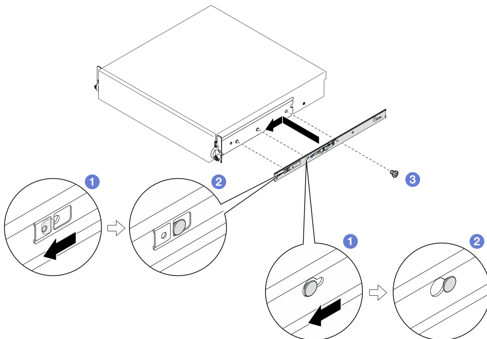
图 16. 安装内侧导轨
