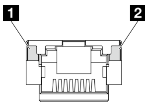
图 231. XCC 系统管理端口 LED
