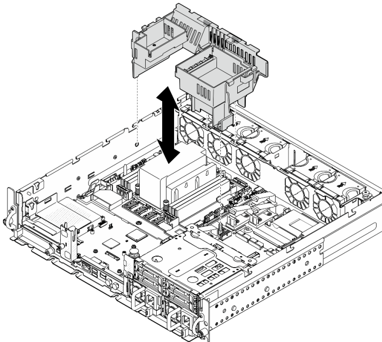
图 37. 为 2U 散热器安装导风罩
