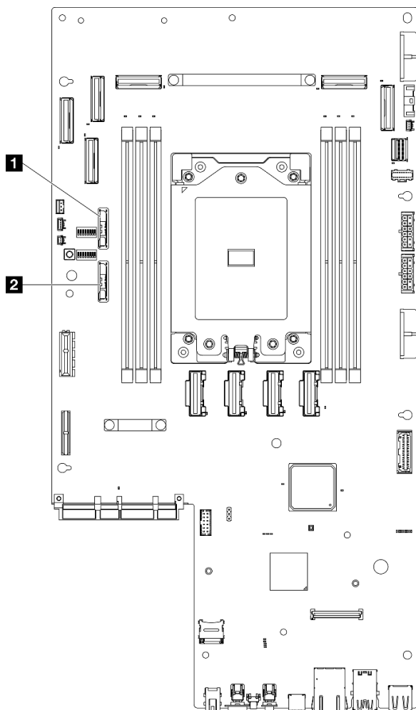
图 46. 主板上的 CMOS 电池位置
