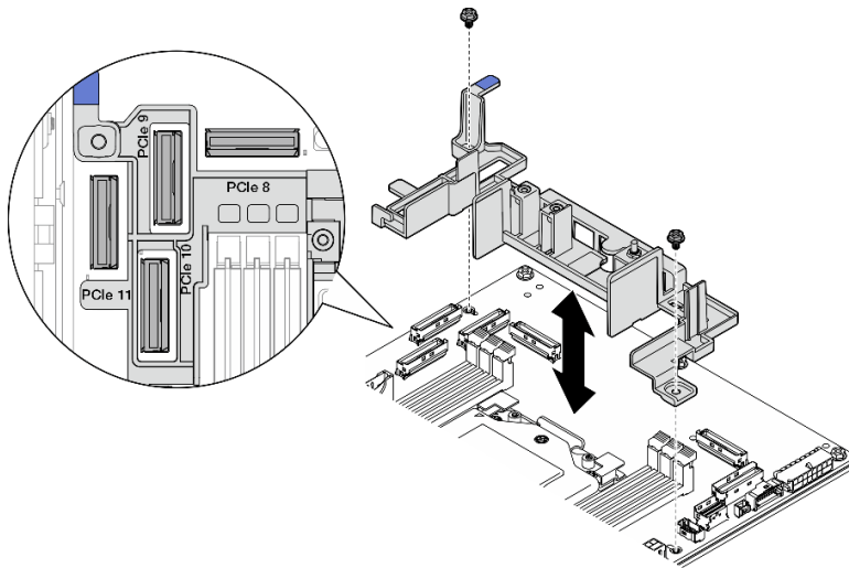
图 43. 安装线缆壁挂支架
