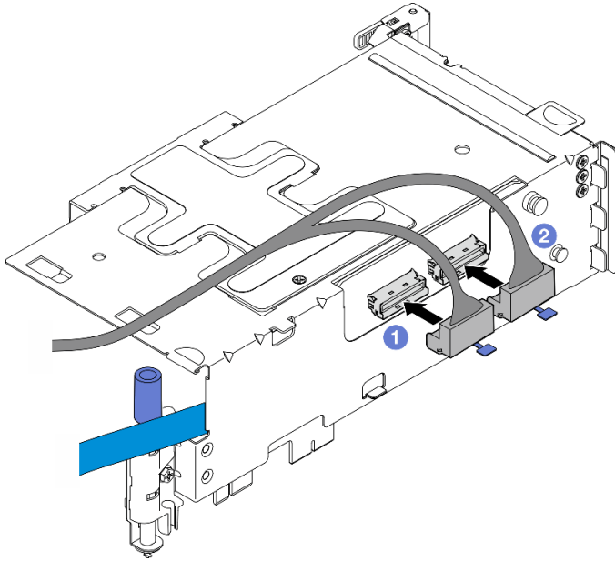
图 146. PCIe 转接卡 1 线缆布放
