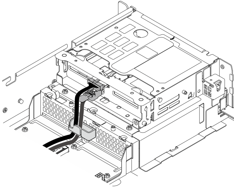
图 60. 正面硬盘背板线缆布放
