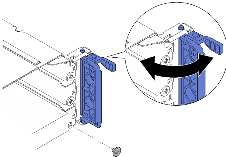
图 183. 安装固定螺钉
