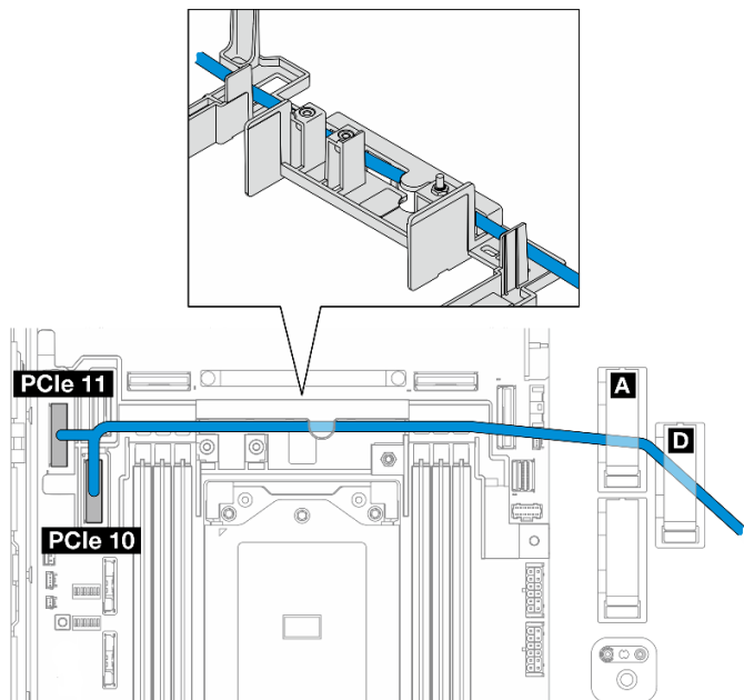
图 217. 正面背板信号线缆
