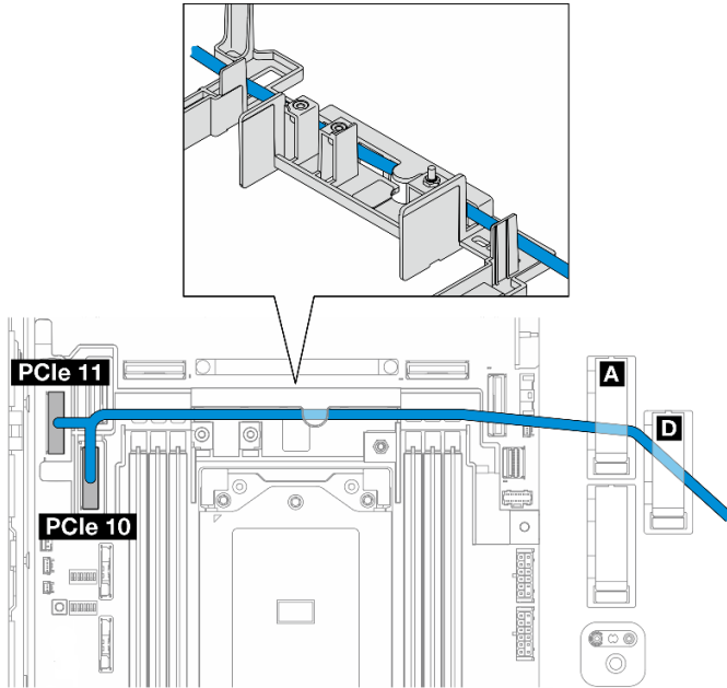
图 220. 正面背板信号线缆
