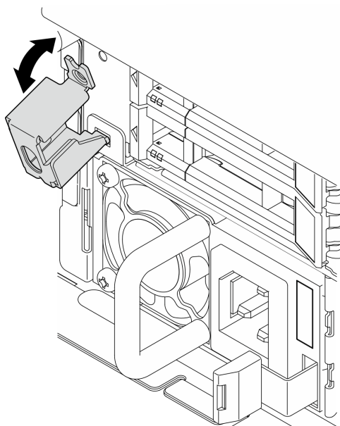
图 177. 卸下安全挡板钥匙锁支架
