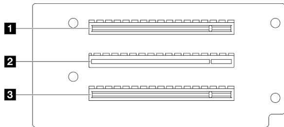
图 201. PCIe 转接卡 2 转接卡
