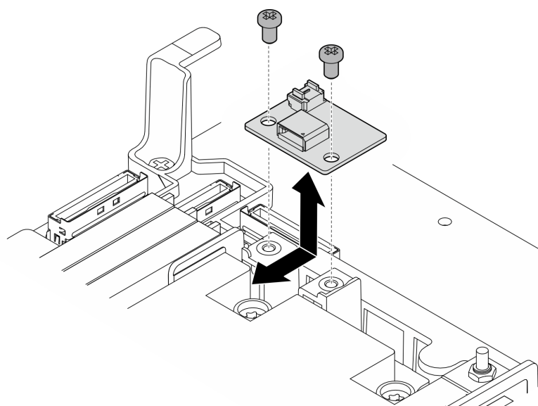
图 39. 安装气流传感器板
