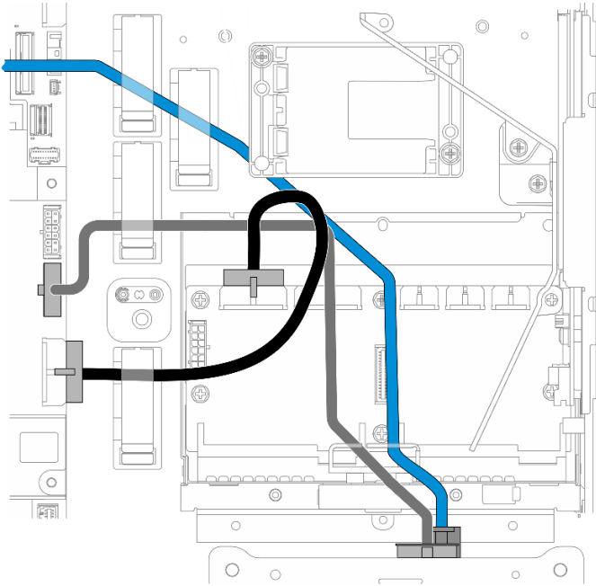
图 225. 正面硬盘背板线缆布放
