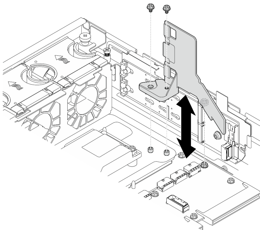
图 29. 为带有内置硬盘仓的配置安装 M.2 导风罩
