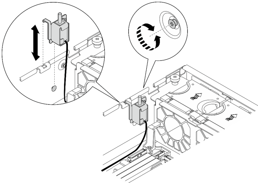
图 79. 卸下入侵感应开关及线缆
