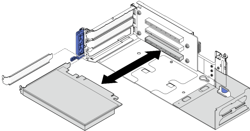
图 119. 从 PCIe 转接卡 2 上卸下 PCIe 适配器
