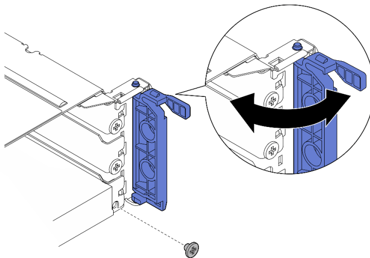
图 126. 安装固定螺钉
