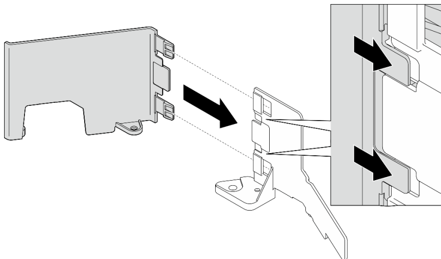
图 28. 组合 M.2 导风罩的前后两部分
