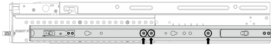
图 10. ThinkEdge 1000 毫米摩擦导轨套件 v2 的内侧导轨有三颗螺钉
