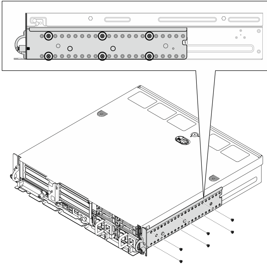
图 14. EIA 支架常规深度 1 到 6: 六颗螺钉
