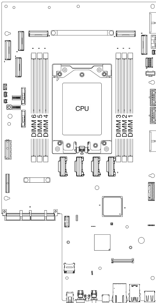
图 1. 内存条和处理器布局
