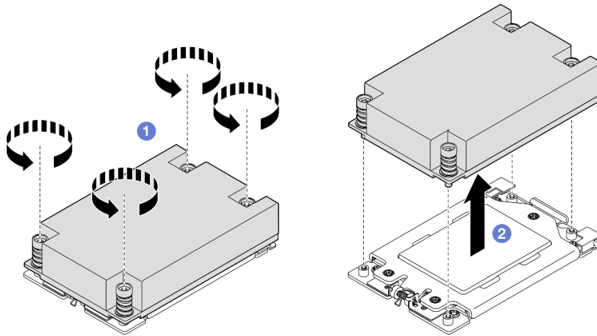
图 156. 卸下 1U 散热器
