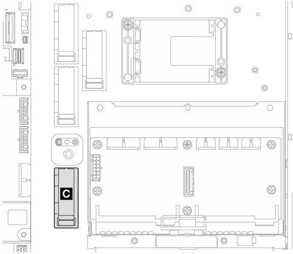
图 221. 线缆夹 C
