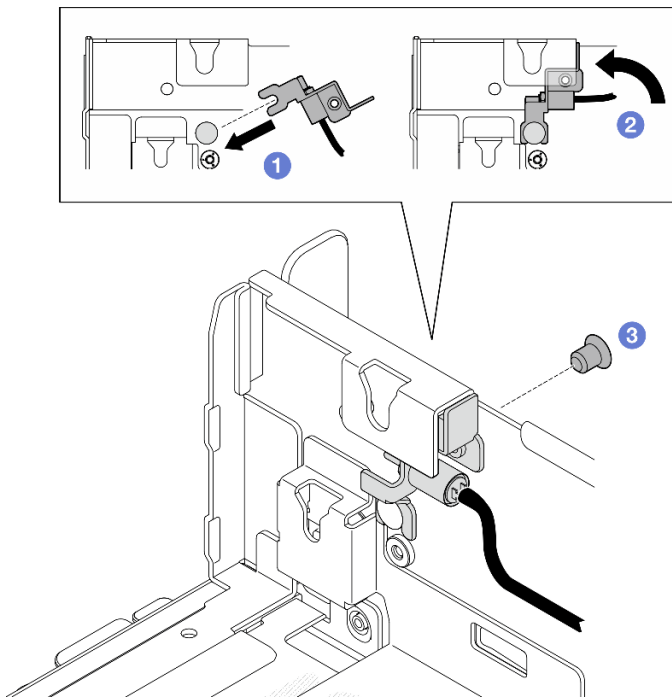
图 41. 安装挡板检测开关
