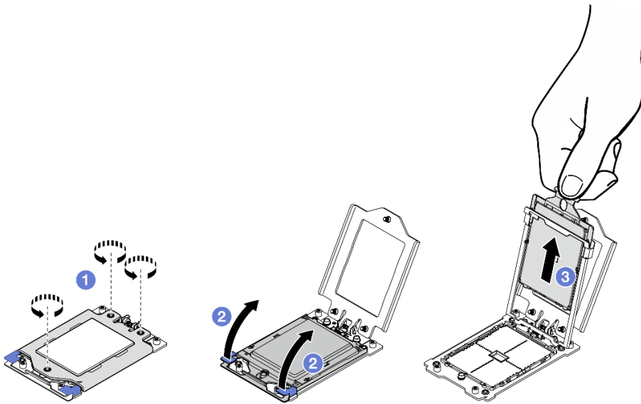
图 158. 卸下处理器
