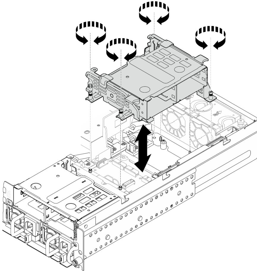
图 70. 安装内置硬盘仓
