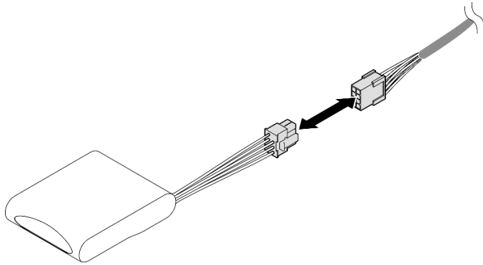
图 167. 断开与延长线缆的连接
