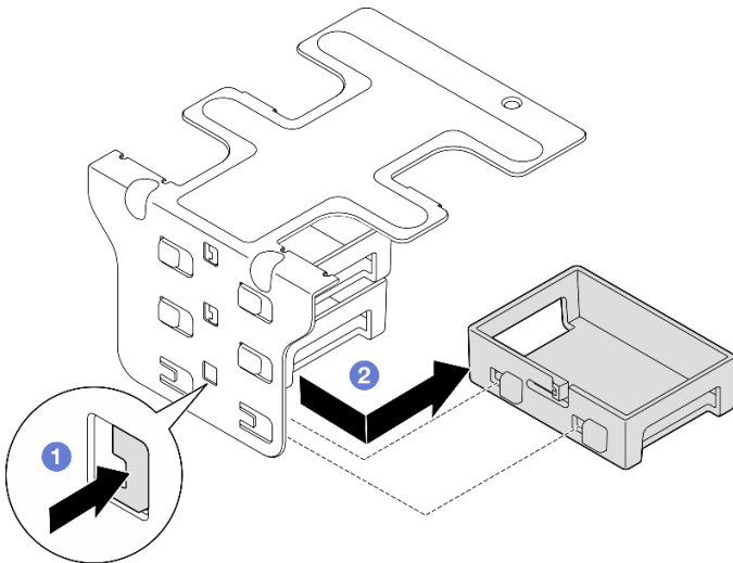
图 116. 卸下半高型填充件
