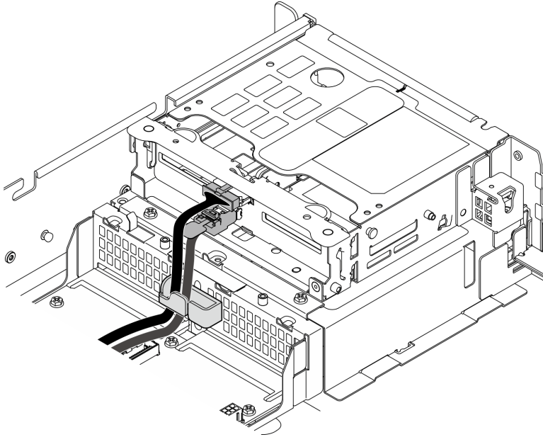
图 224. 正面硬盘背板线缆布放
