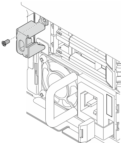
图 176. 卸下安全挡板钥匙锁支架
