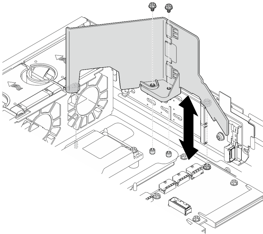
图 30. 为不带内置硬盘仓的配置安装 M.2 导风罩
