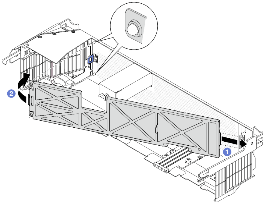
图 173. 安装灰尘过滤器
