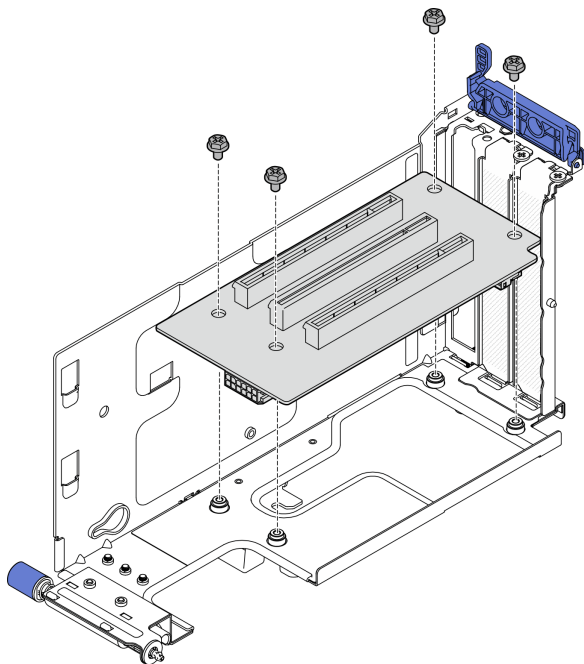
图 147. 安装转接卡
