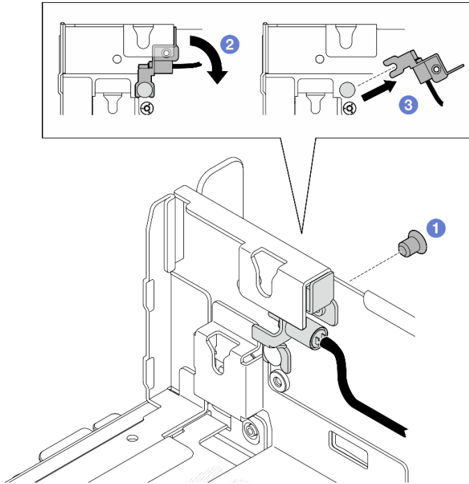
图 40. 卸下挡板检测开关
