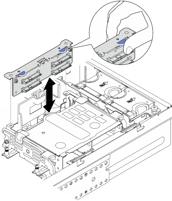
图 111. 卸下内置硬盘背板
