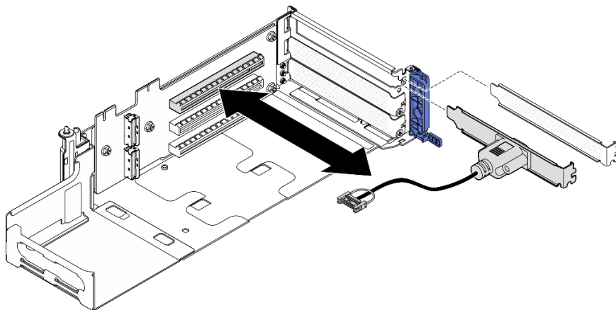
图 181. 卸下串口模块
