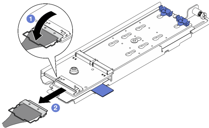
图 83. 从 SATA/NVMe M.2 背板上断开线缆
