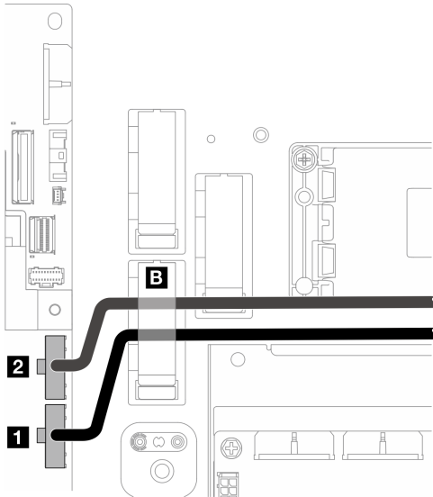
图 213. 背板电源线
