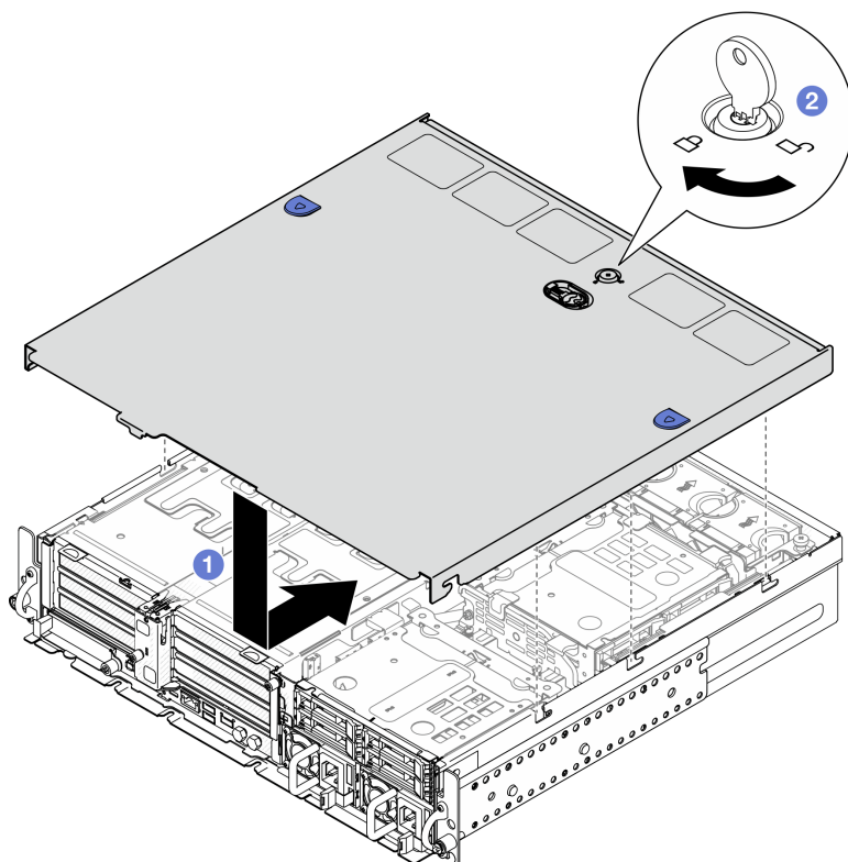
图 193. 安装顶盖
