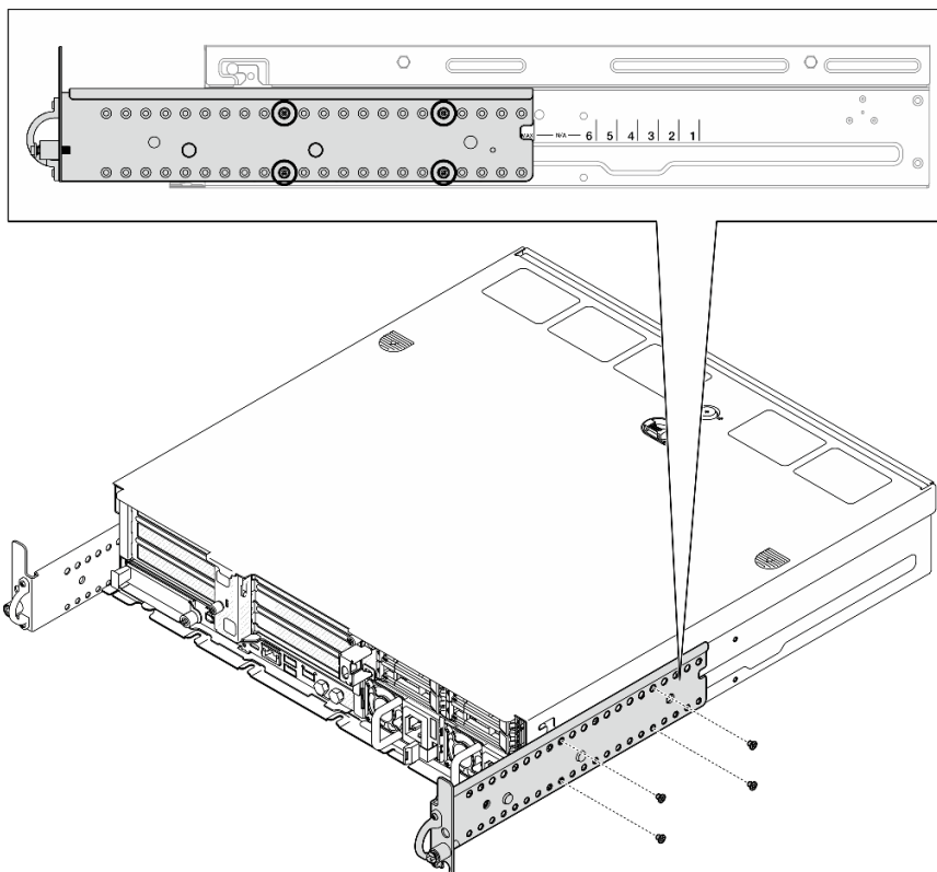
图 15. 用于安全挡板的 EIA 支架最大深度：四颗螺钉
