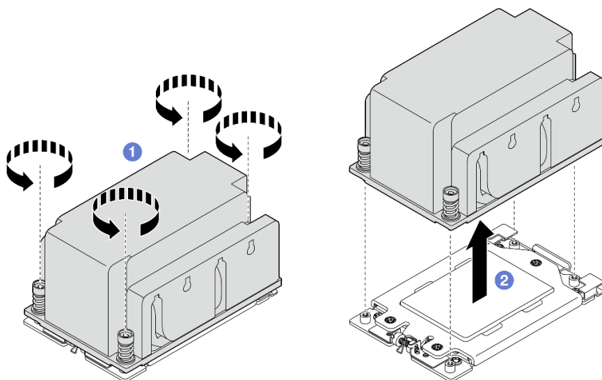
图 157. 卸下 2U 散热器
