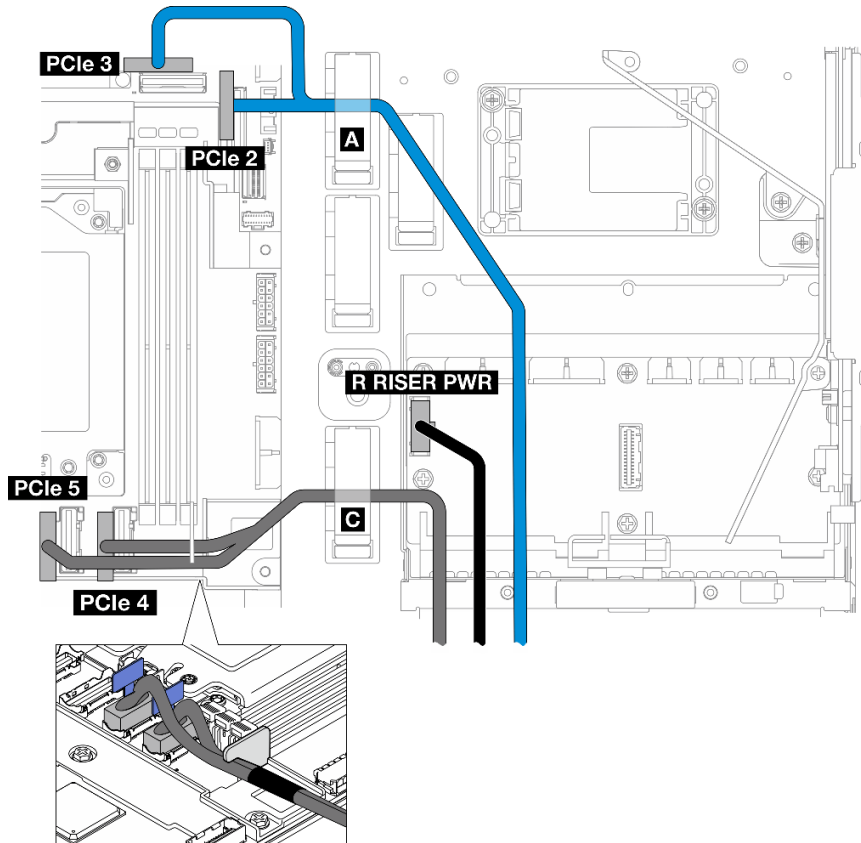
图 209. PCIe 转接卡 2 线缆布放
