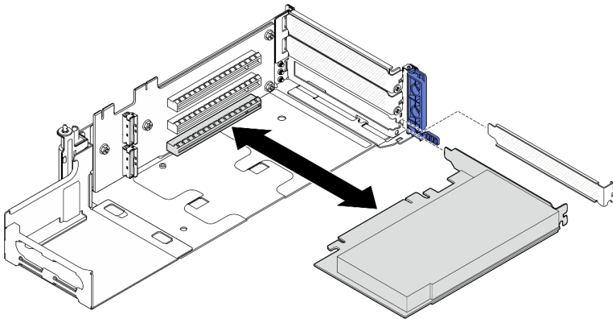
图 124. 将 PCIe 适配器安装到 PCIe 转接卡 1 上
