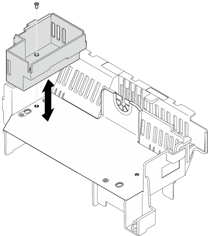
图 33. 更换转接卡 1 填充件
