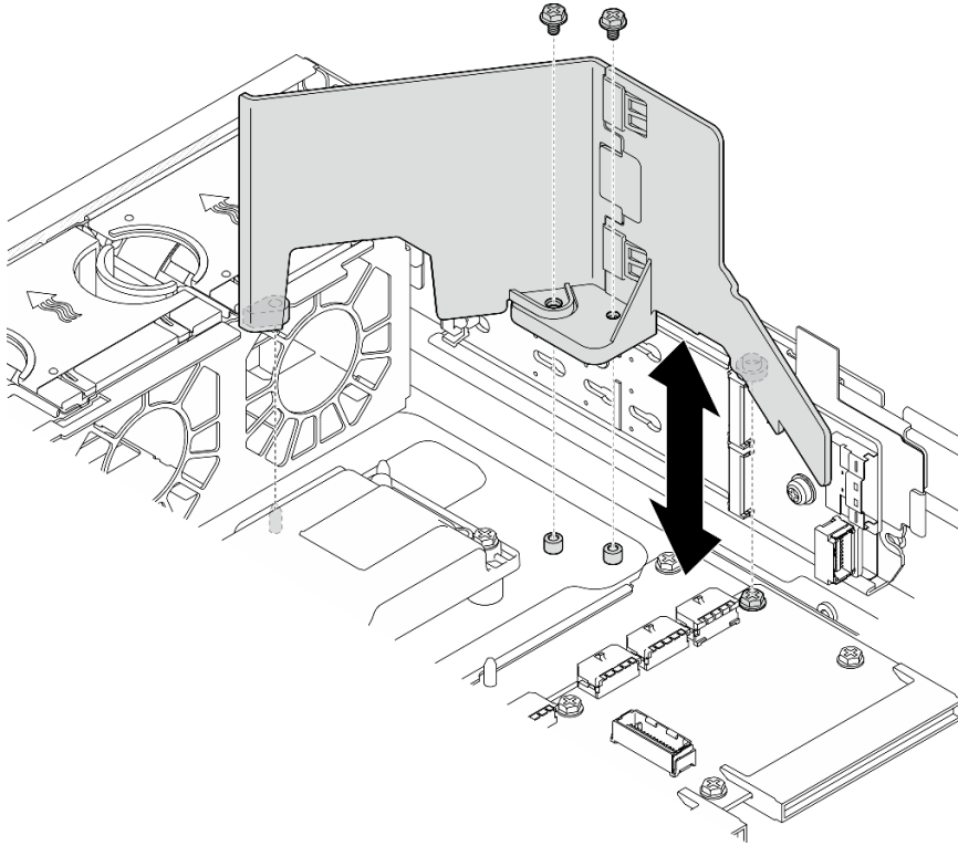
图 26. 为不带内置硬盘仓的配置卸下 M.2 导风罩
