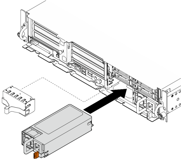
图 155. 安装电源模块单元
