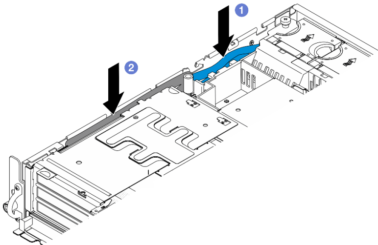
图 133. 整理 PCIe 转接卡 1 信号线缆
