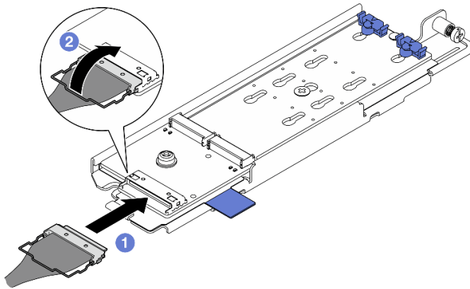
图 94. 将线缆连接到 SATA/NVMe M.2 背板
