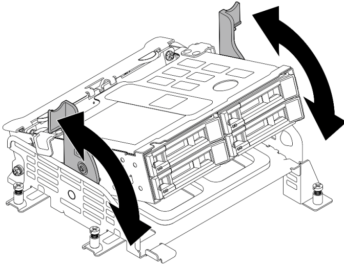
图 78. 转动内置硬盘仓
