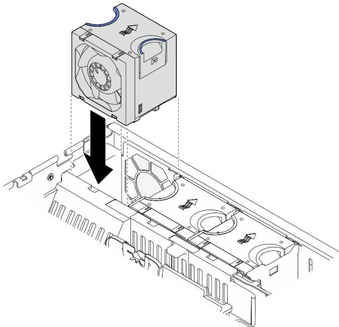
图 49. 安装风扇
