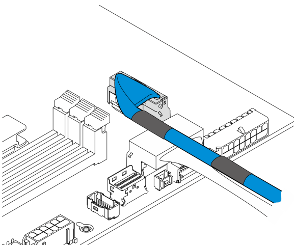
图 219. 内置背板信号线缆
