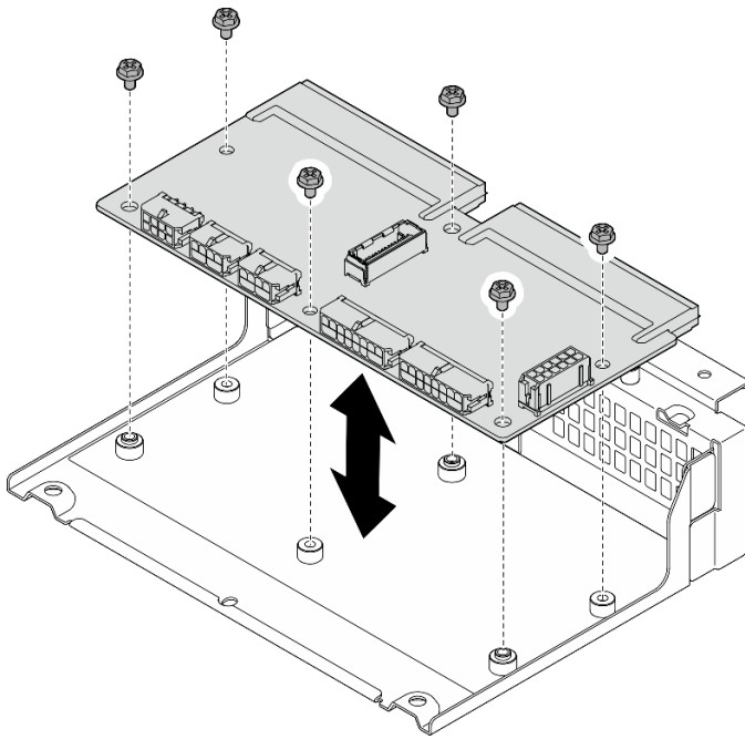
图 153. 安装配电板
