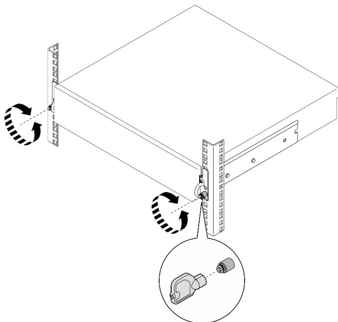
图 3. 将服务器与机架分离：安全 EIA 支架
