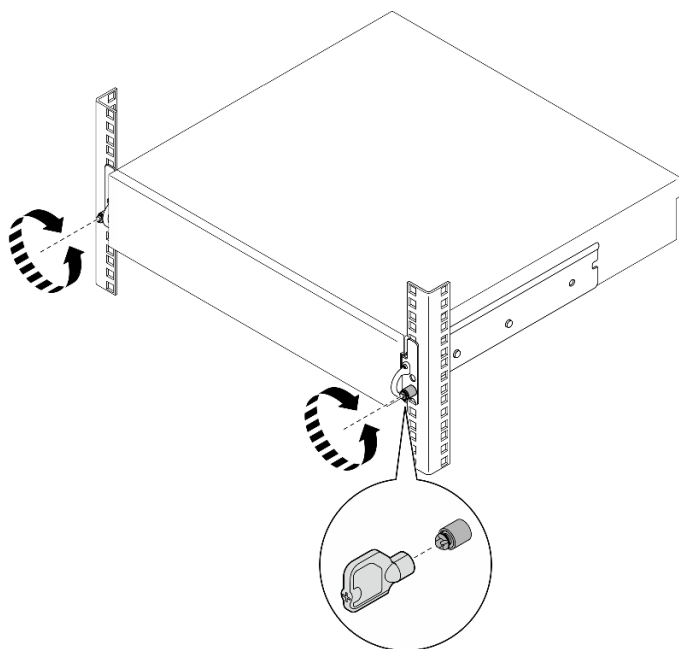
图 24. 将服务器固定到机架：安全 EIA 支架
