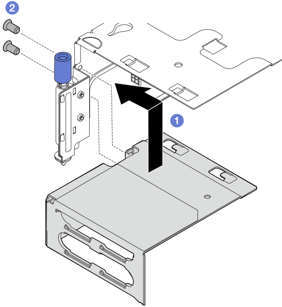
图 123. 将扩展器安装到 PCIe 转接卡 2
