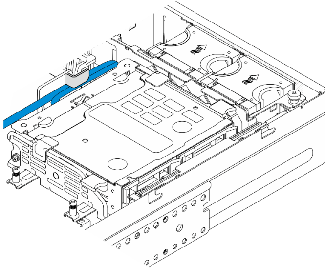
图 74. 内置硬盘背板线缆布放
