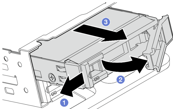
图 64. 卸下内置硬盘
