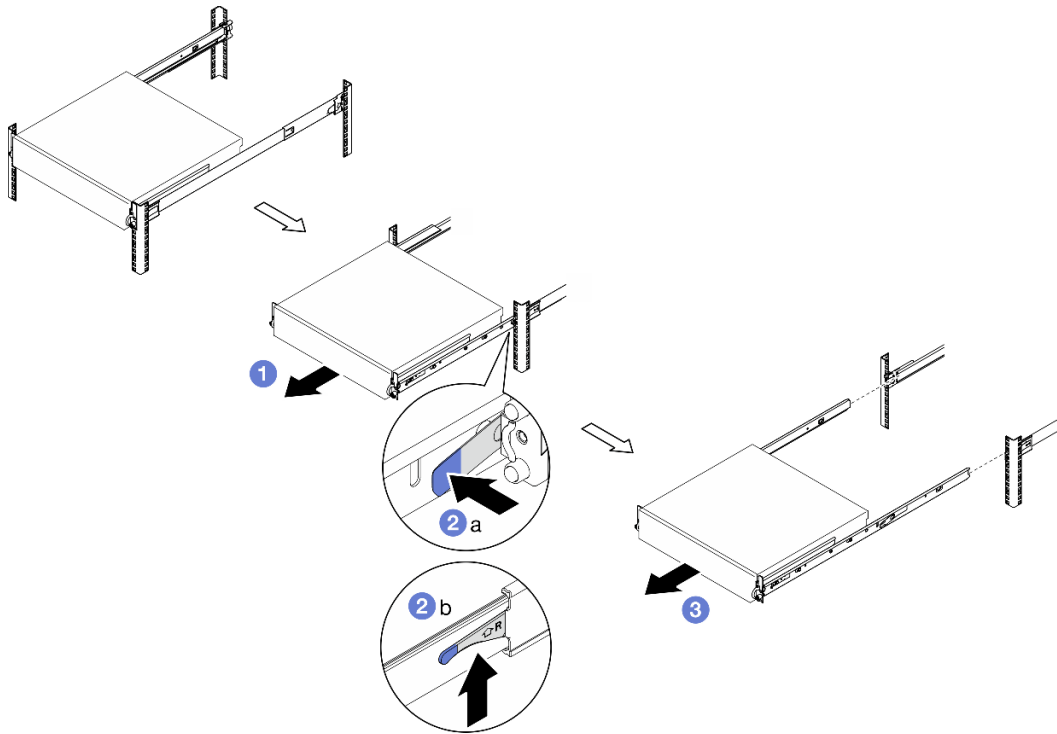
图 4. 从机架上卸下服务器
