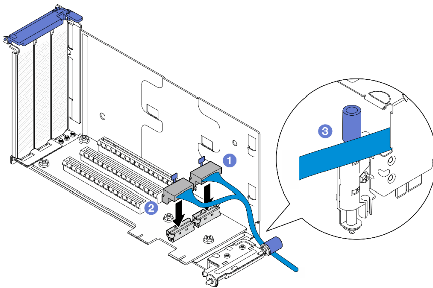
图 145. PCIe 转接卡 1 线缆布放
