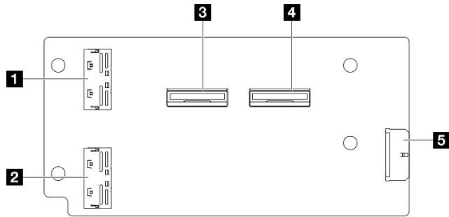
图 200. PCIe 转接卡 2 转接卡
