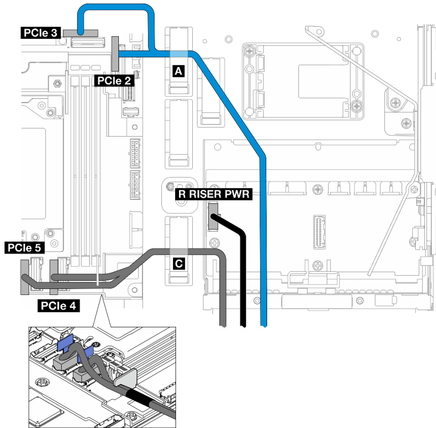
图 136. PCIe 转接卡 2 线缆布放
