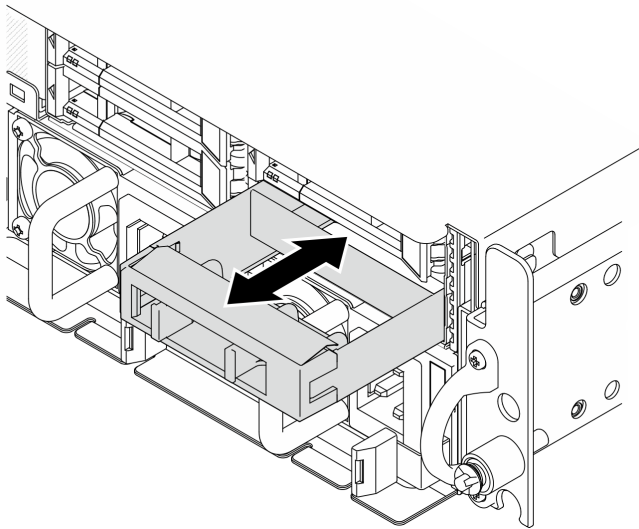
图 61. 卸下硬盘填充件
