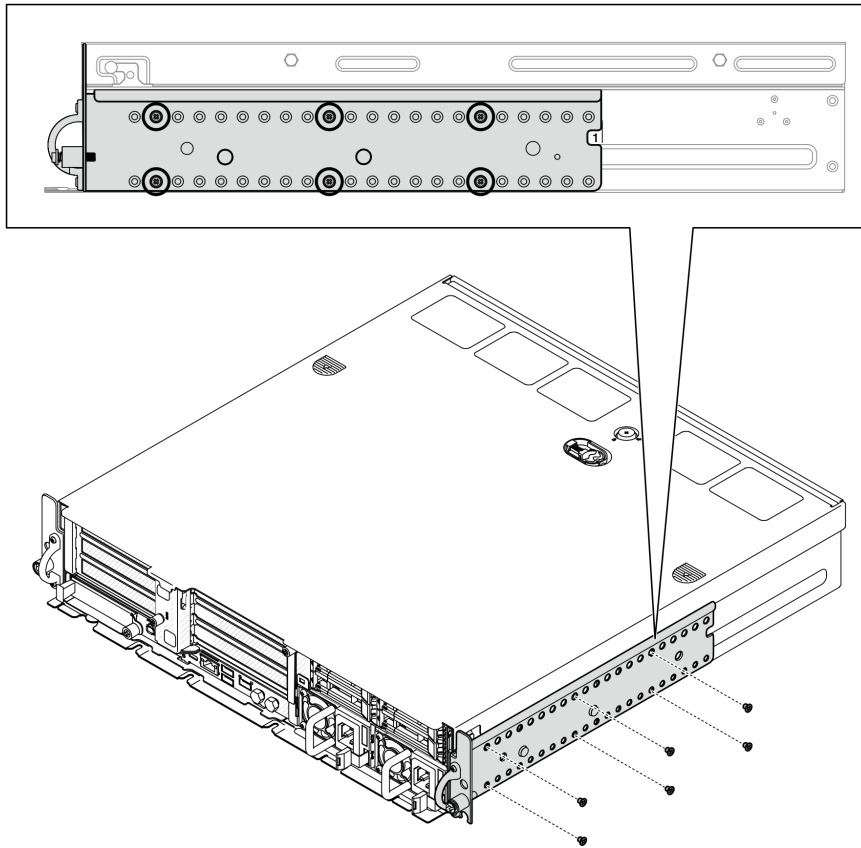
图 11. EIA 支架常规深度 1 到 6: 六颗螺钉
