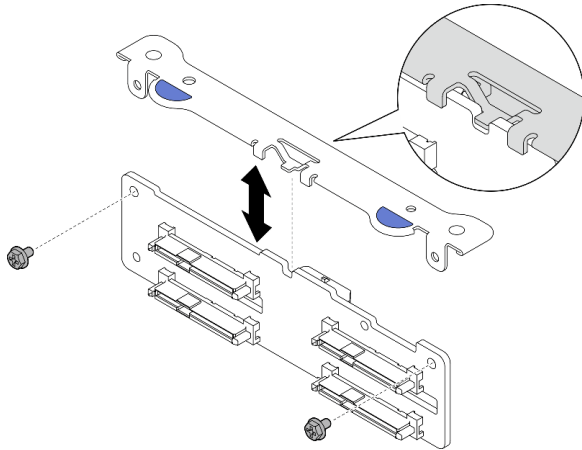
图 58. 将背板固定到背板支架
