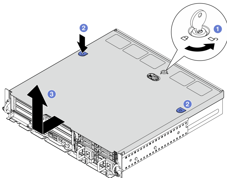
图 192. 卸下顶盖
