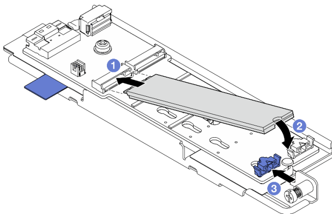
图 92. 安装 M.2 硬盘
