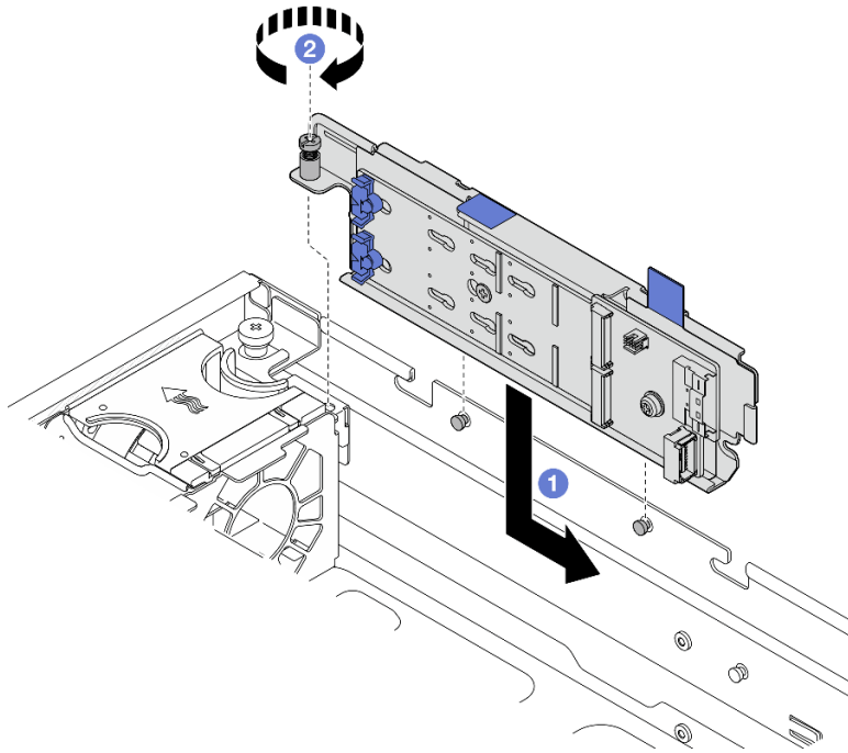
图 95. 安装 M.2 背板组合件
