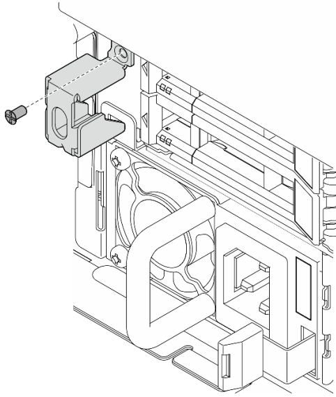
图 179. 安装安全挡板钥匙锁支架
