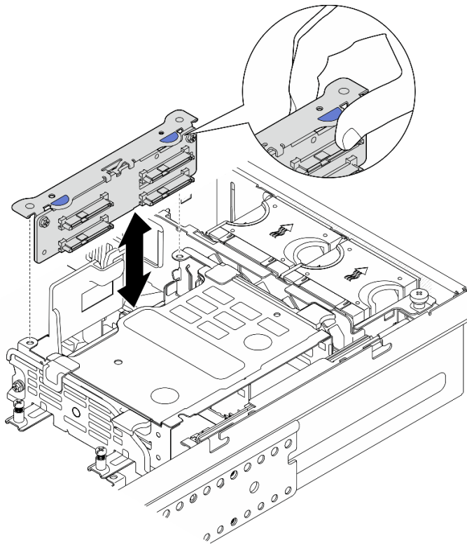
图 73. 安装内置硬盘背板
