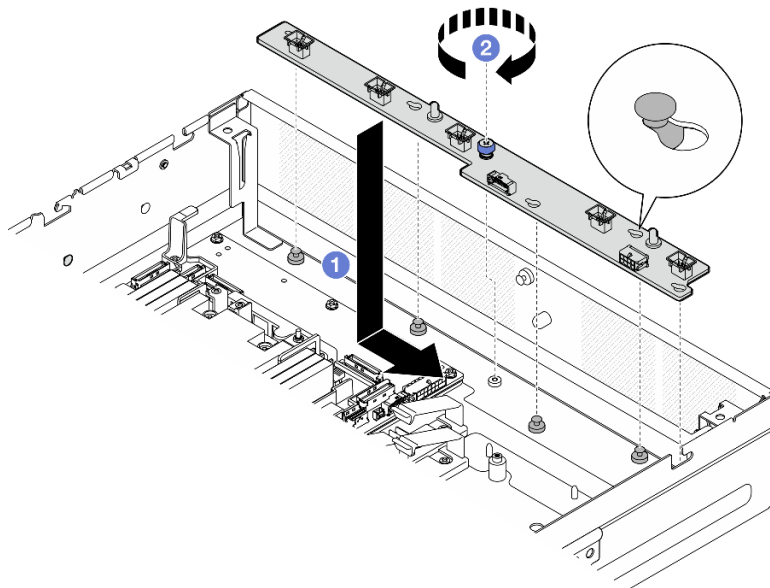
图 52. 安装风扇控制板
