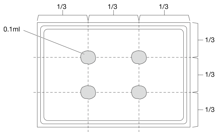
图 160. 涂抹导热油脂
