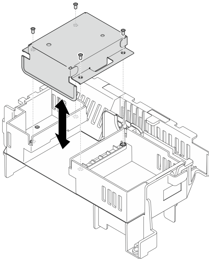
图 35. 更换中间填充件
