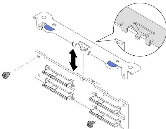
图 67. 从背板支架上拆下硬盘背板
