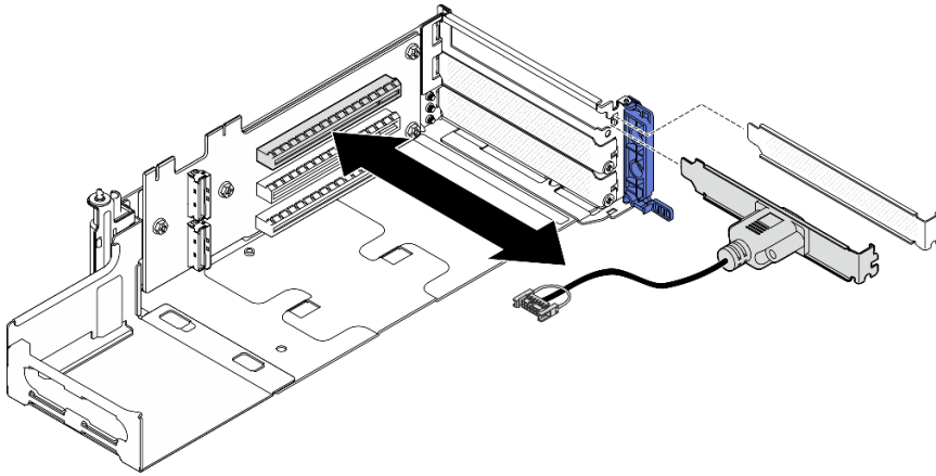
图 182. 安装串口模块
