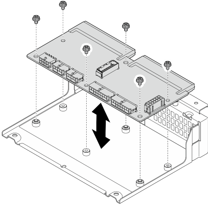
图 150. 卸下配电板
