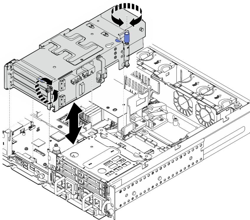
图 137. 安装 PCIe 转接卡 2
