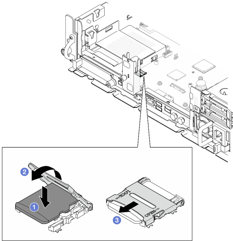
图 101. 安装 MicroSD 卡
