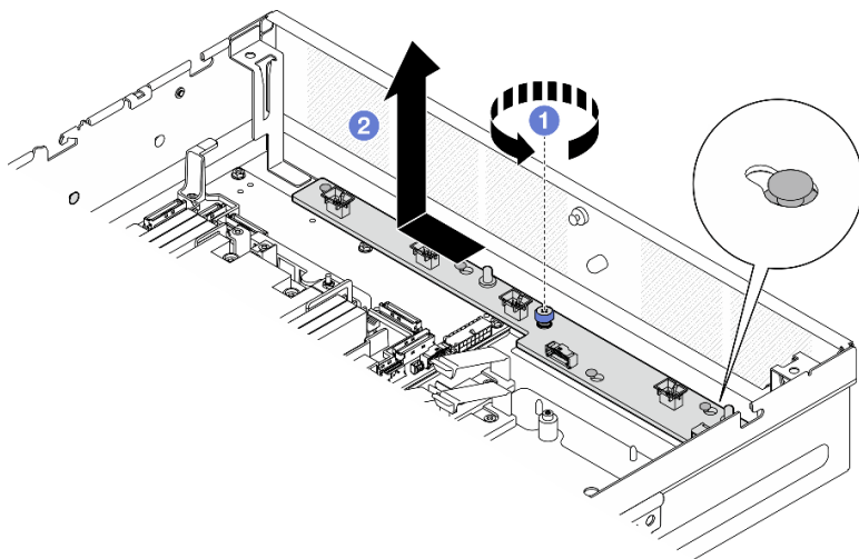
图 51. 卸下风扇控制板
