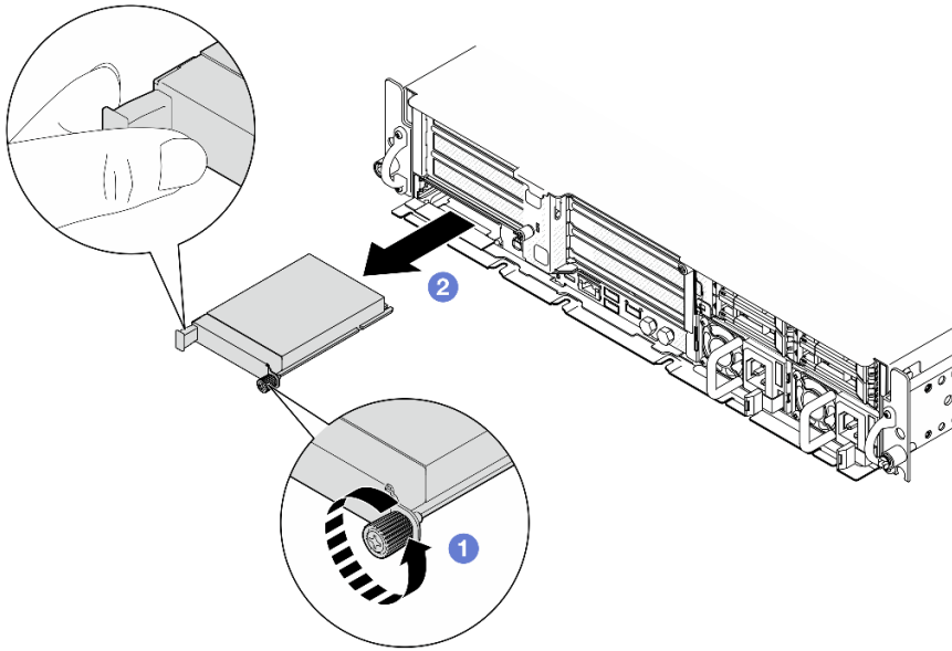
图 102. 卸下 OCP 模块
