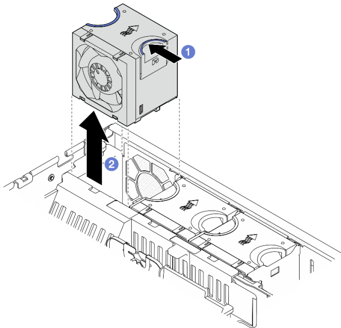
图 48. 卸下风扇模块
