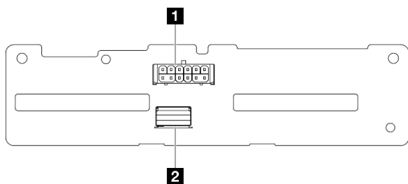
图 194. SAS/SATA 背板接口
