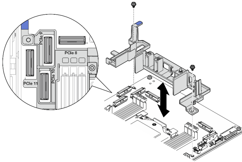
图 42. 卸下线缆壁挂支架
