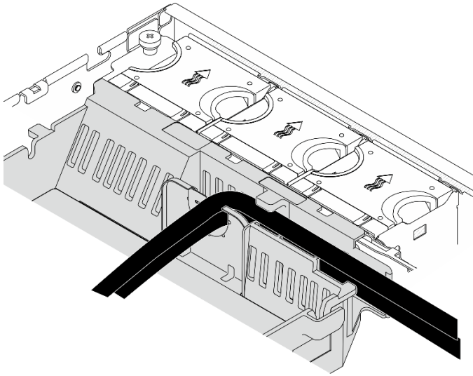
图 134. 处理器导风罩上的 GPU 电源线
