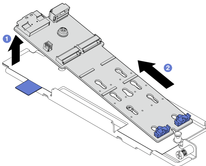
图 87. 卸下 M.2 背板
