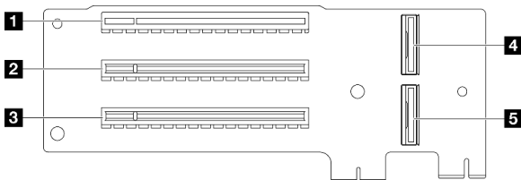
图 199. PCIe 转接卡 1 转接卡
