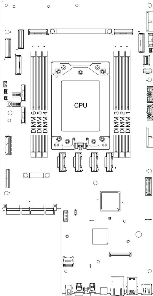
图 98. 内存条和处理器布局
