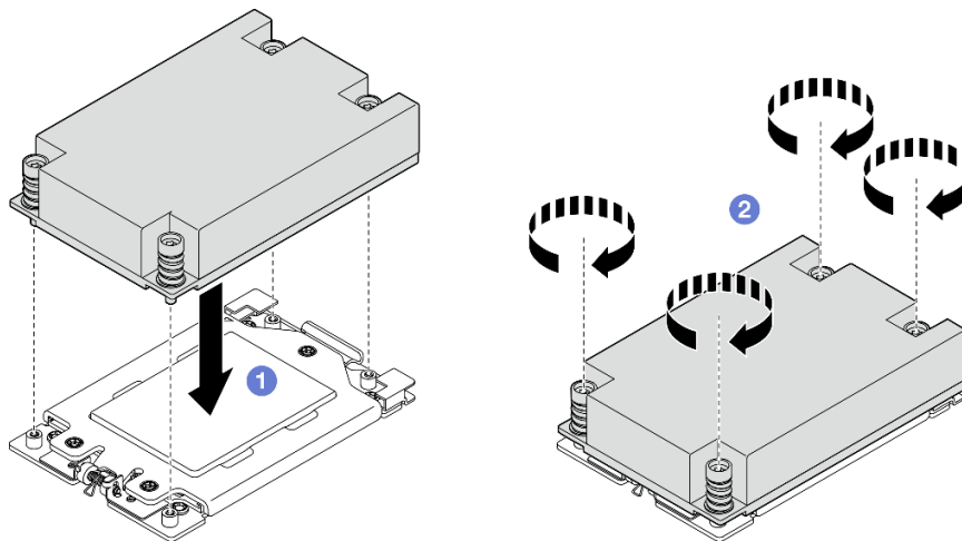
图 161. 安装 1U 散热器
