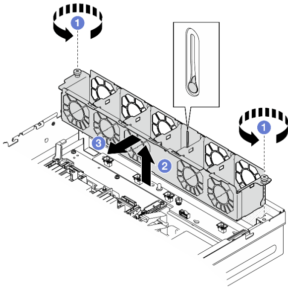
图 50. 卸下风扇架
