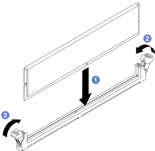
图 99. 安装内存条
