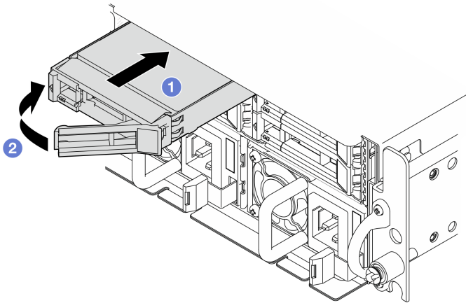
图 62. 安装正面热插拔硬盘
