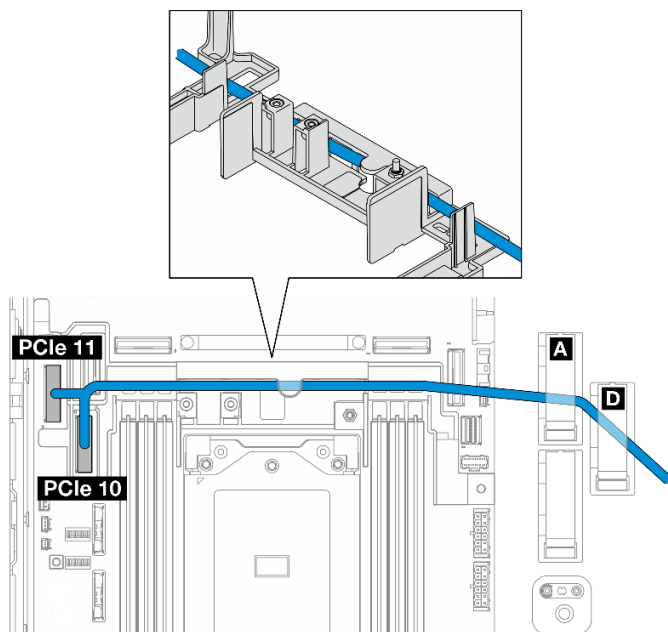
图 222. 正面背板信号线缆
