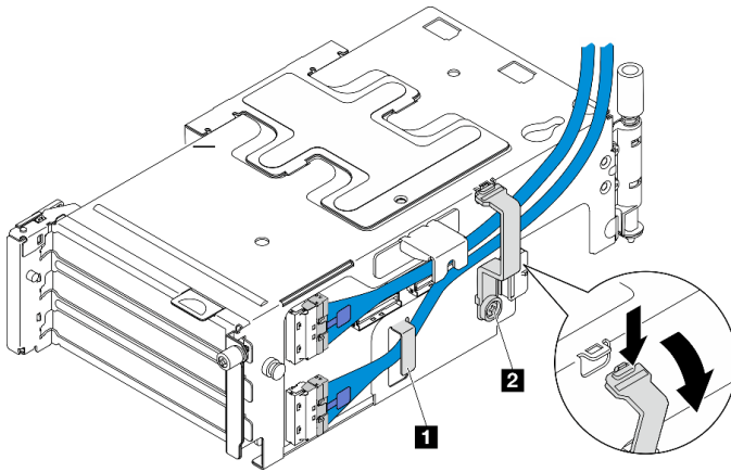
图 141. PCIe 转接卡 2 线缆布放
