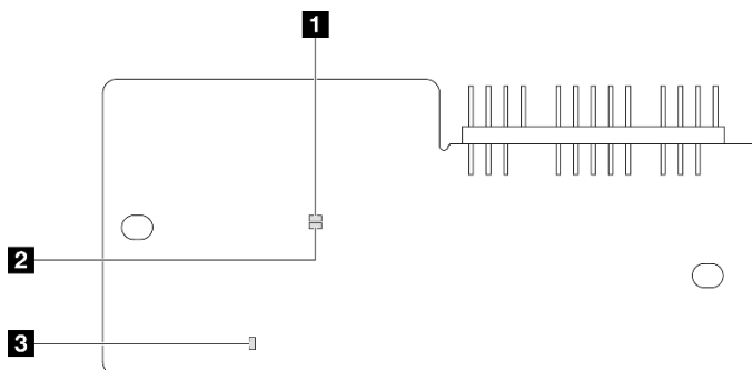
图 234. 固件和 RoT 安全模块上的 LED
