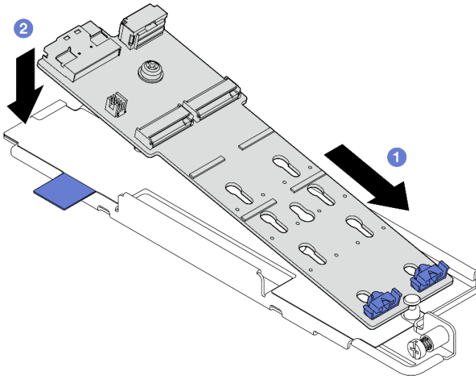
图 88. 安装 M.2 背板
