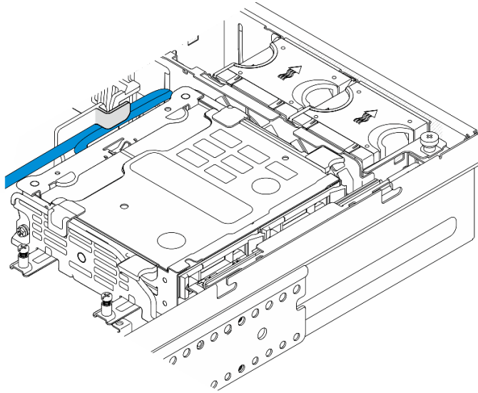
图 140. 整理线缆
