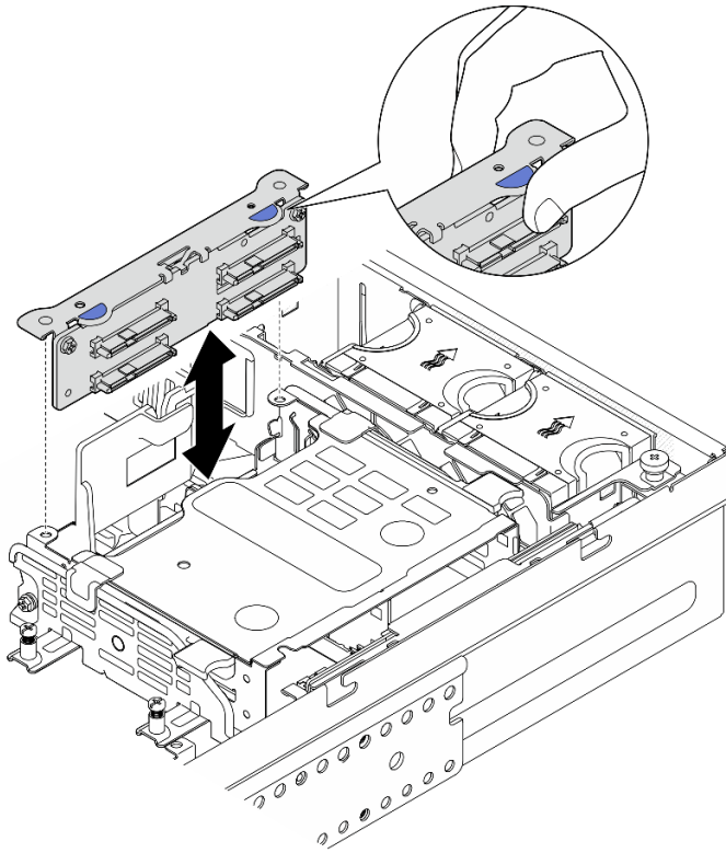
图 139. 安装内置硬盘背板
