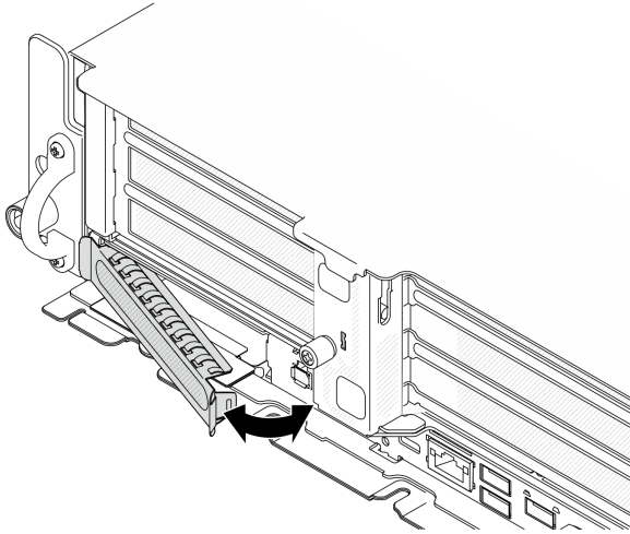
图 104. 卸下 OCP 填充件
