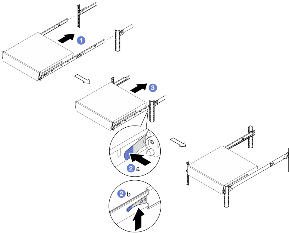
图 22. 将服务器安装到机架
