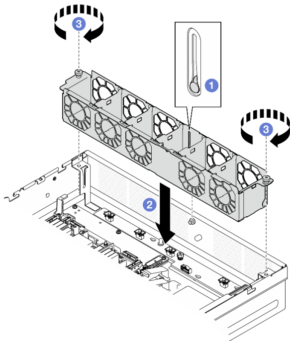
图 53. 安装风扇架
