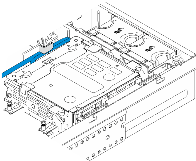
图 65. 由处理器导风罩的线缆夹固定的线缆
