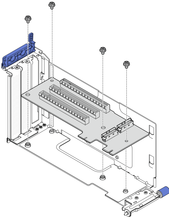
图 144. 安装转接卡
