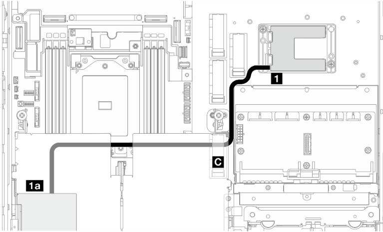
图 211. PCIe 转接卡 1 上的 RAID 适配器
