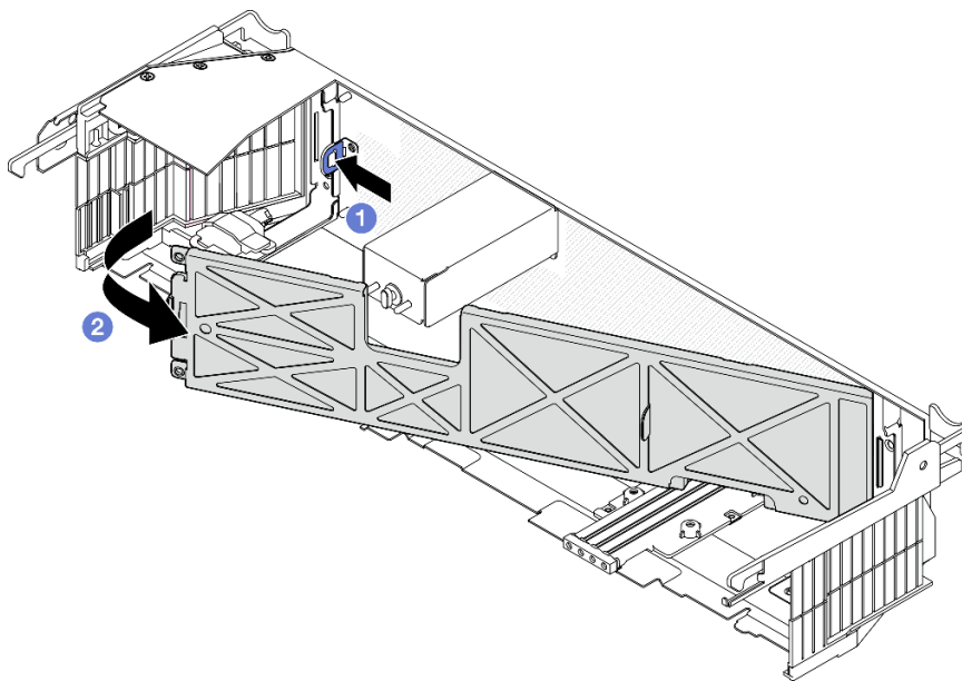
图 172. 卸下灰尘过滤器
