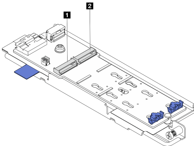
图 84. M.2 硬盘插槽编号
