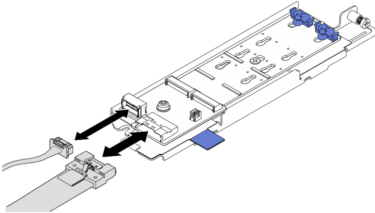
图 93. 将线缆连接到 SATA/x4 NVMe M.2 背板
