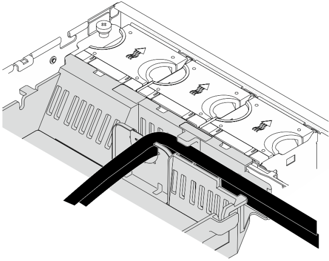
图 106. 处理器导风罩上的 GPU 电源线
