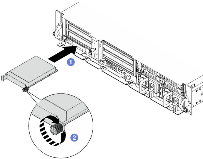
图 105. 安装 OCP 模块
