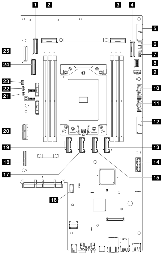
图 202. 主板接口
