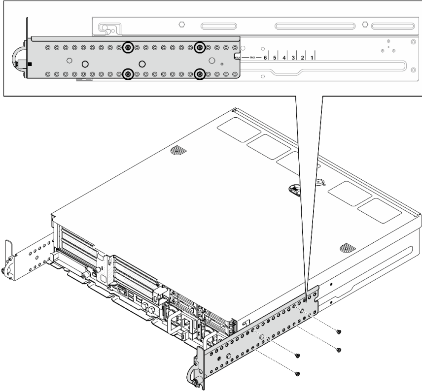
图 12. 用于安全挡板的 EIA 支架最大深度：四颗螺钉
