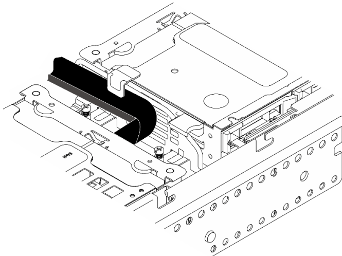
图 75. 正面硬盘背板线缆布放
