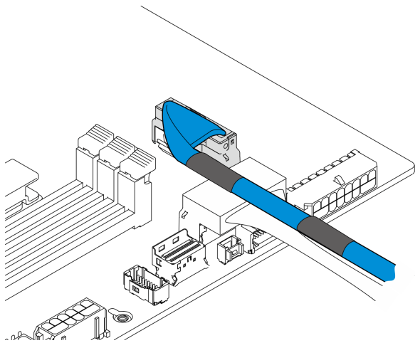
图 216. 内置背板信号线缆
