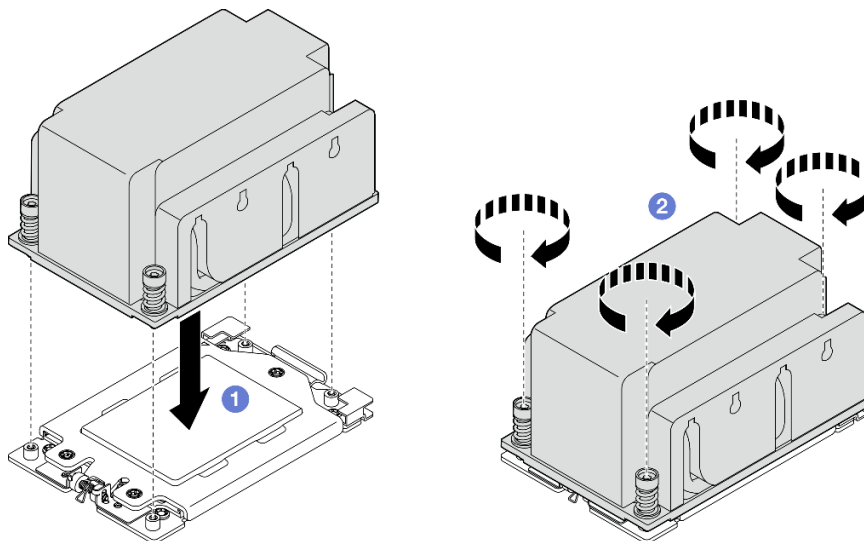
图 162. 安装 2U 散热器
