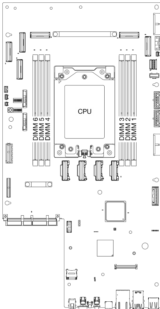
图 96. 内存条和处理器布局
