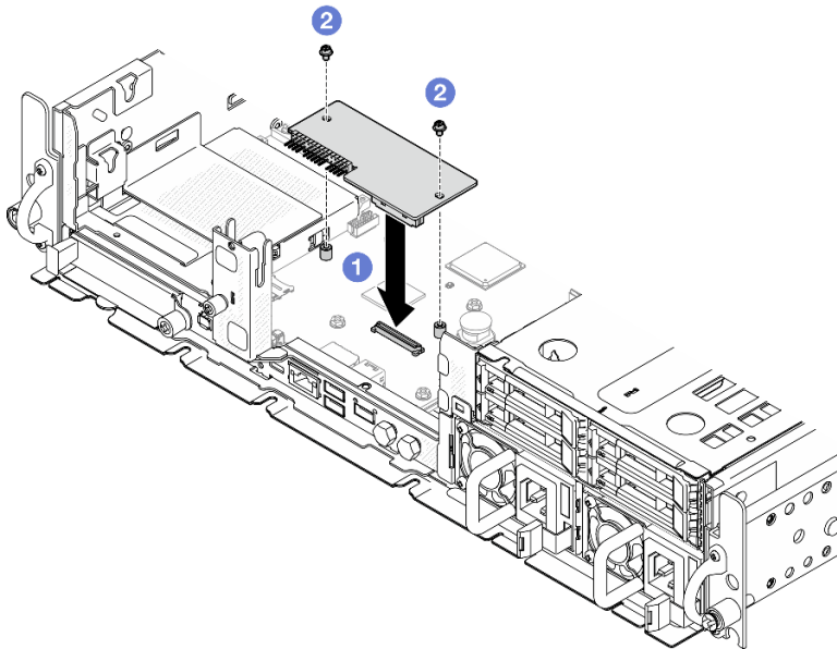
图 185. 安装固件和 RoT 安全模块
