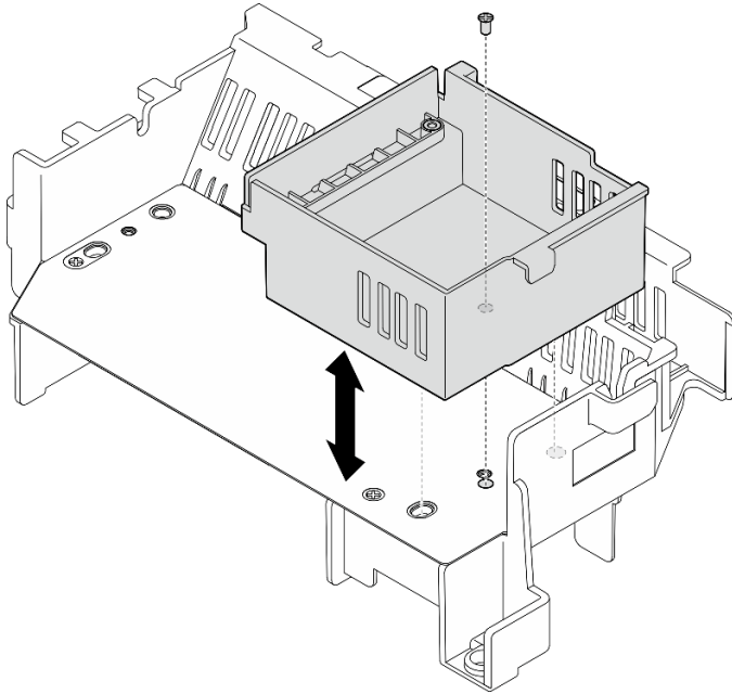
图 34. 更换转接卡 2 填充件
