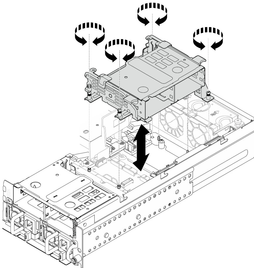
图 68. 卸下内置硬盘仓
