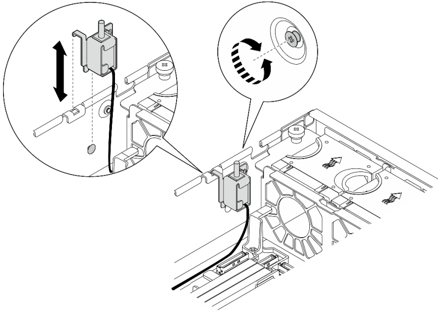
图 80. 安装入侵感应开关
