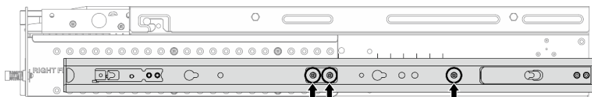
图 21. ThinkEdge 1000 毫米摩擦导轨套件 v2 的 inner 导轨有三颗螺钉
