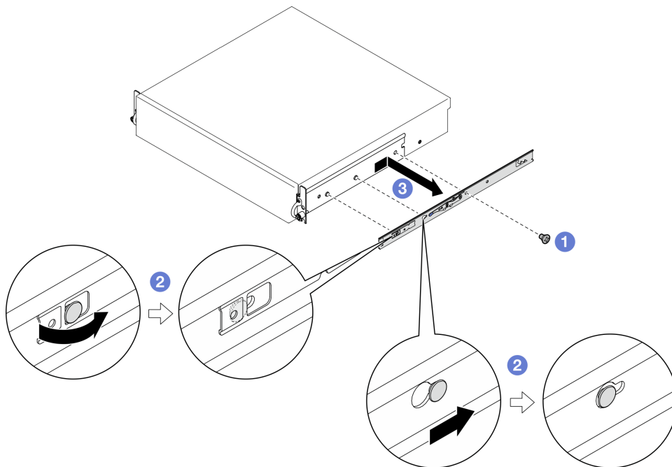
图 5. 卸下内侧导轨
