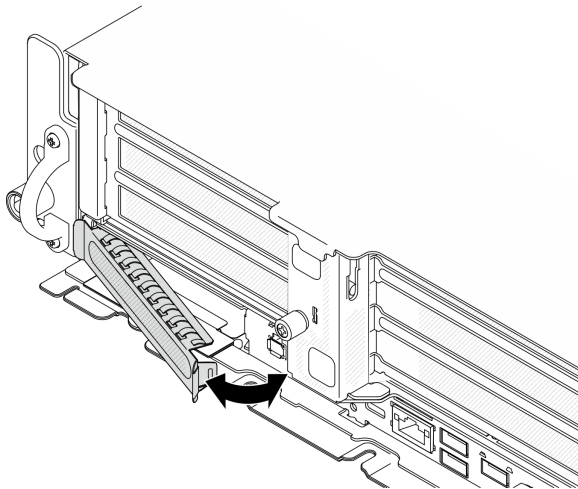
图 103. 安装 OCP 填充件
