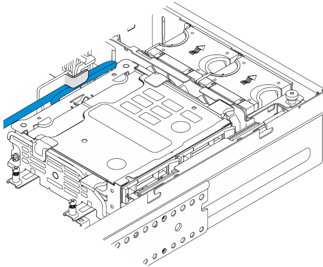
图 110. 由处理器导风罩的线缆夹固定的线缆
