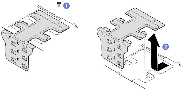
图 115. 卸下侧面支架
