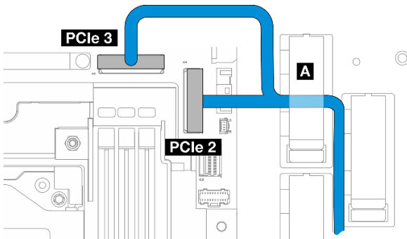
图 218. 内置背板信号线缆
