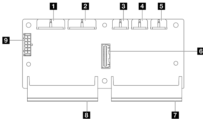
图 197. 配电板接口
