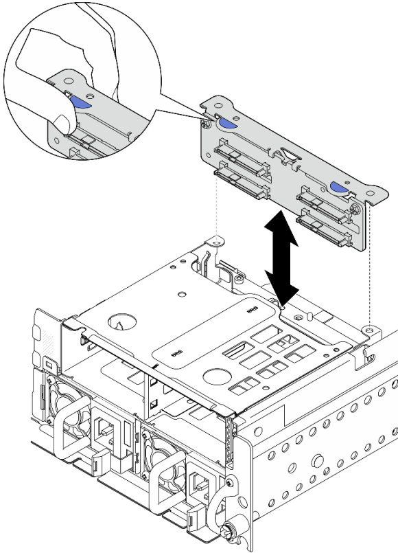
图 56. 卸下正面硬盘背板
