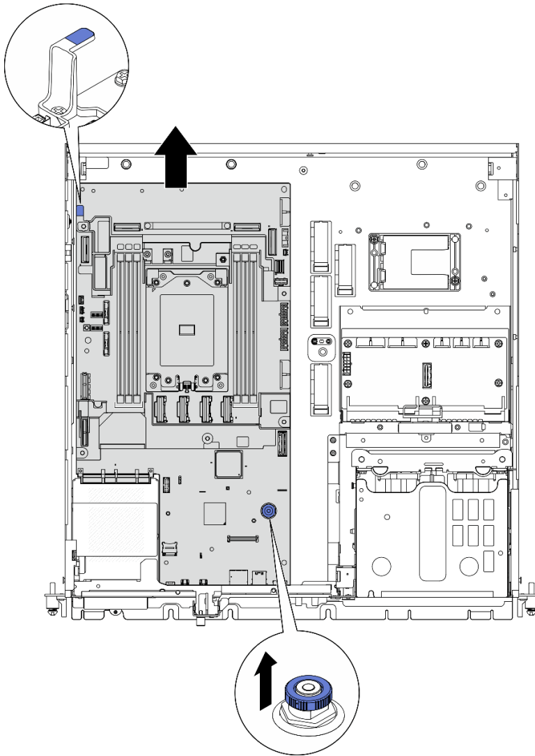
图 186. 拆卸主板
