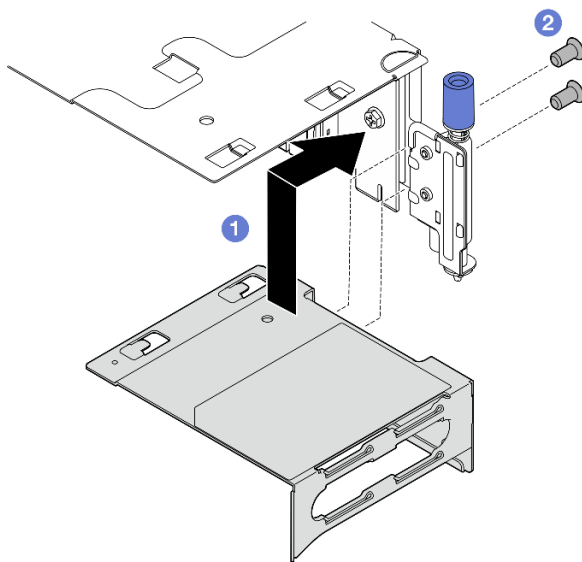
图 122. 将扩展器安装到 PCIe 转接卡 1
