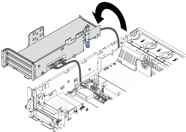
图 109. 将 PCIe 转接卡 1 放在机箱旁边
