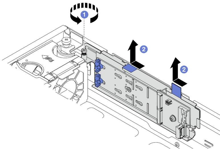
图 81. 卸下 M.2 背板组合件
