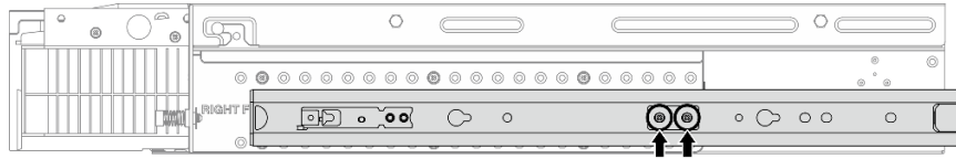
图 9. ThinkEdge 1000 毫米摩擦导轨套件 v2 的内侧导轨有两颗螺钉
