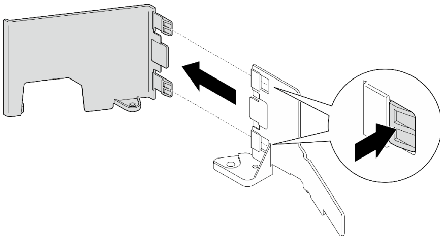
图 27. 将 M.2 导风罩的前后两部分分开
