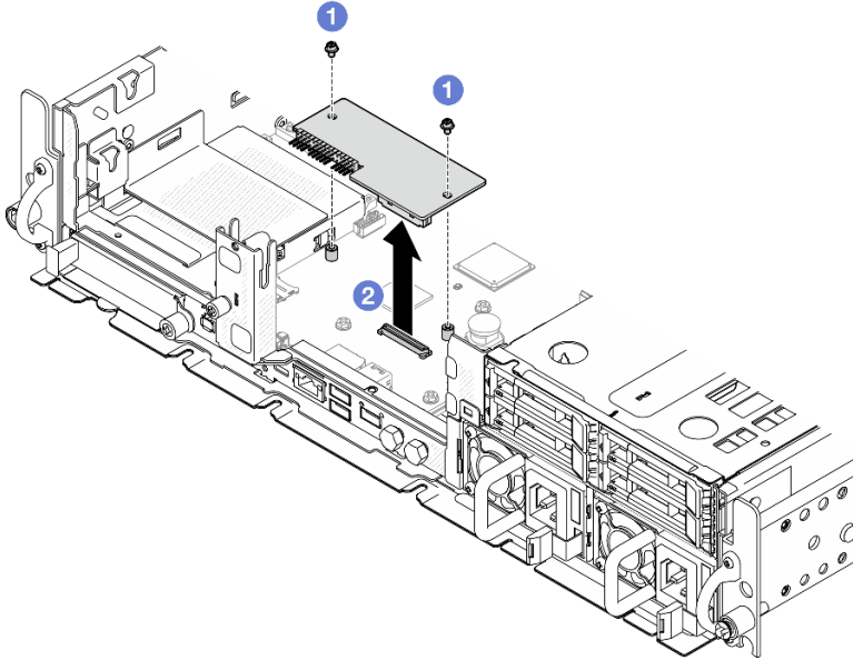
图 184. 卸下固件和 RoT 安全模块
