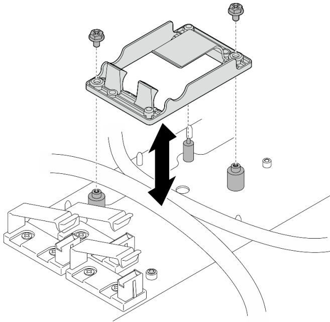
图 169. 安装 RAID 快速充电模块夹持器
