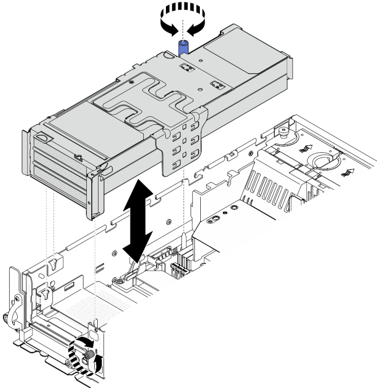
图 108. 提起 PCIe 转接卡 1
