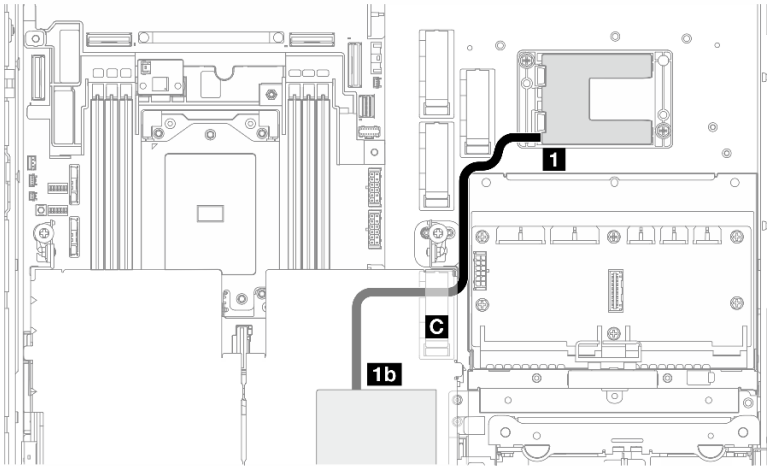
图 212. PCIe 转接卡 2 上的 RAID 适配器
