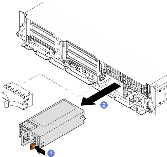
图 154. 卸下电源模块单元
