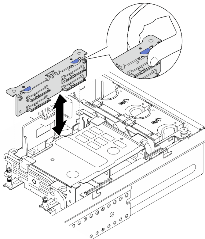
图 66. 卸下内置硬盘背板
