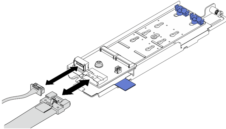
图 82. 从 SATA/x4 NVMe M.2 背板上断开线缆
