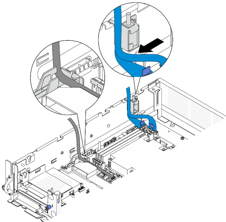
图 208. PCIe 转接卡 1 线缆布放
