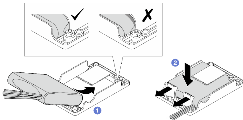
图 166. 安装 RAID 快速充电模块
