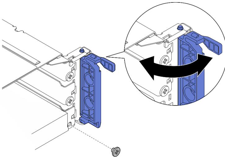
图 180. 卸下固定螺钉
