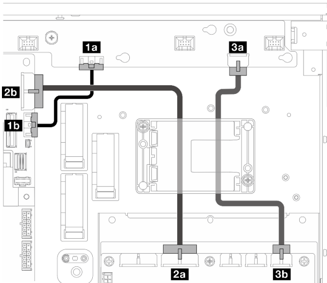
图 203. PDB 和 FCB 线缆布放
