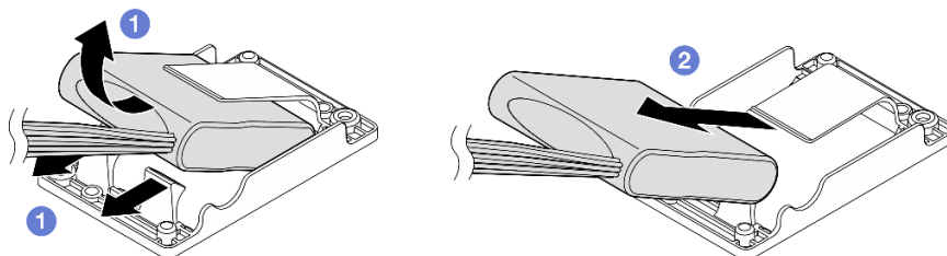
图 163. 卸下 RAID 快速充电模块
