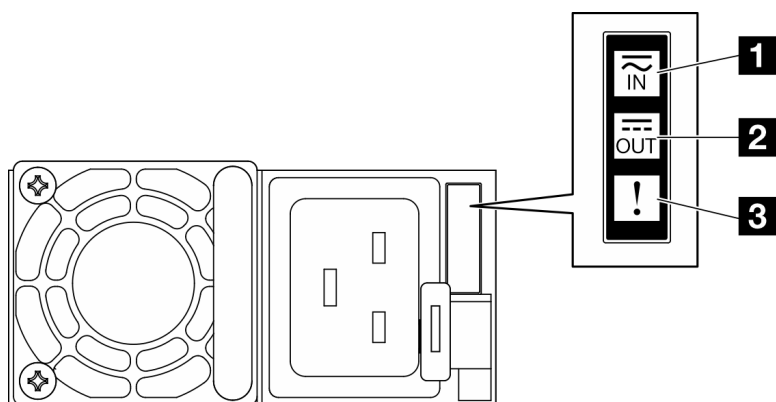
图 232. 电源模块 LED
