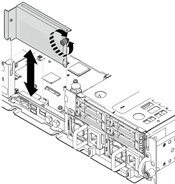
图 135. 卸下转接卡空填充件
