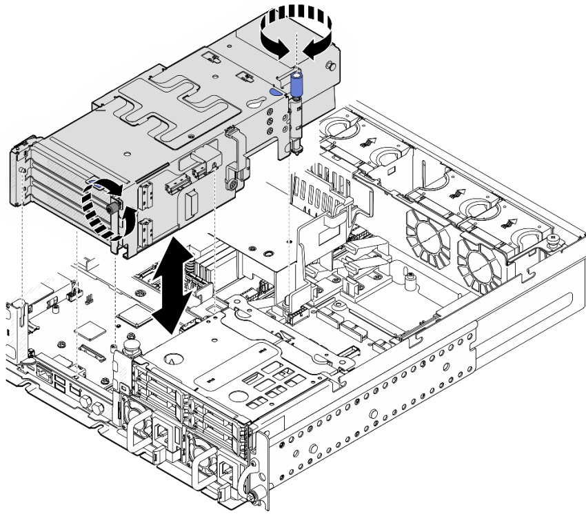
图 113. 提起 PCIe 转接卡 2
