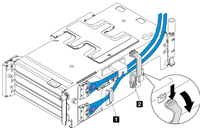
图 148. PCIe 转接卡 2 线缆布放
