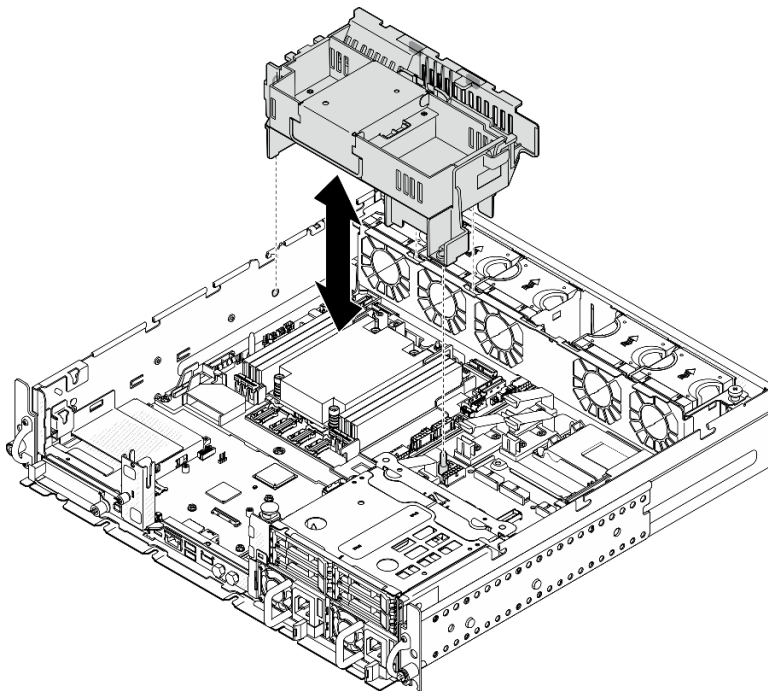
图 31. 为 1U 散热器卸下导风罩
