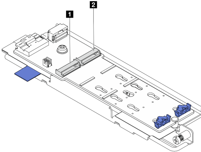
图 91. M.2 硬盘插槽编号
