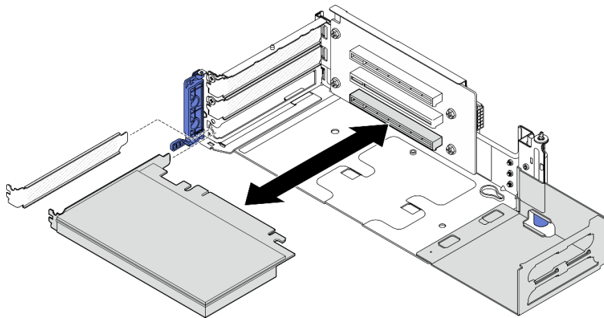
圖例 119. 從 PCIe 擴充卡 2 卸下 PCIe 配接卡
