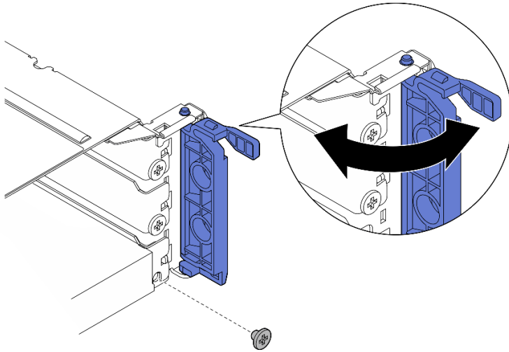
圖例 183. 安裝固定螺絲
