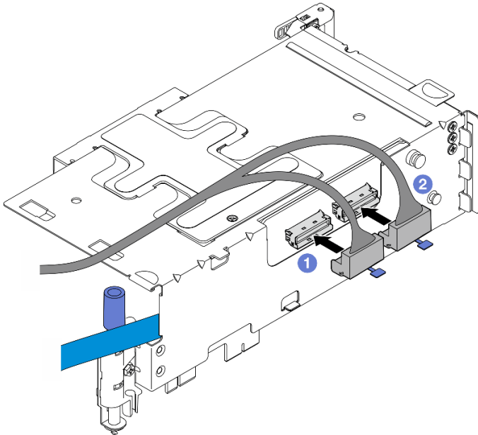
圖例 146. PCIe 擴充卡 1 纜線佈線
