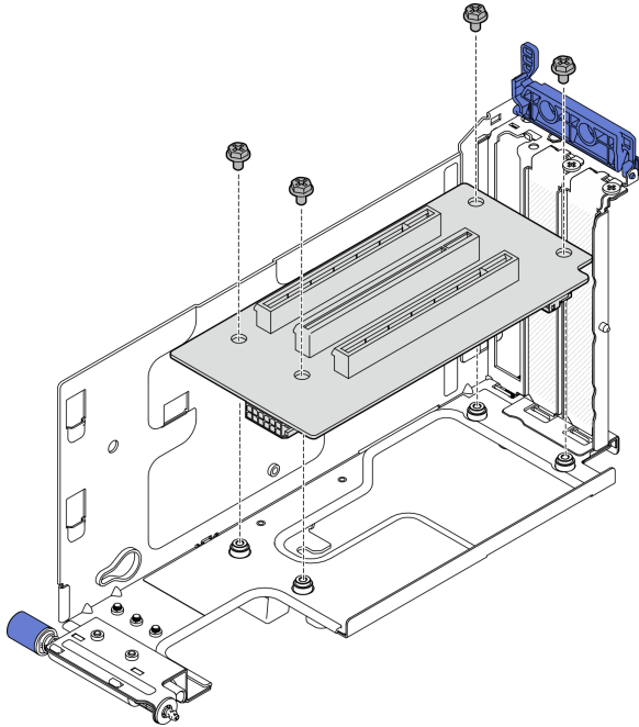
圖例 147. 安裝擴充卡
