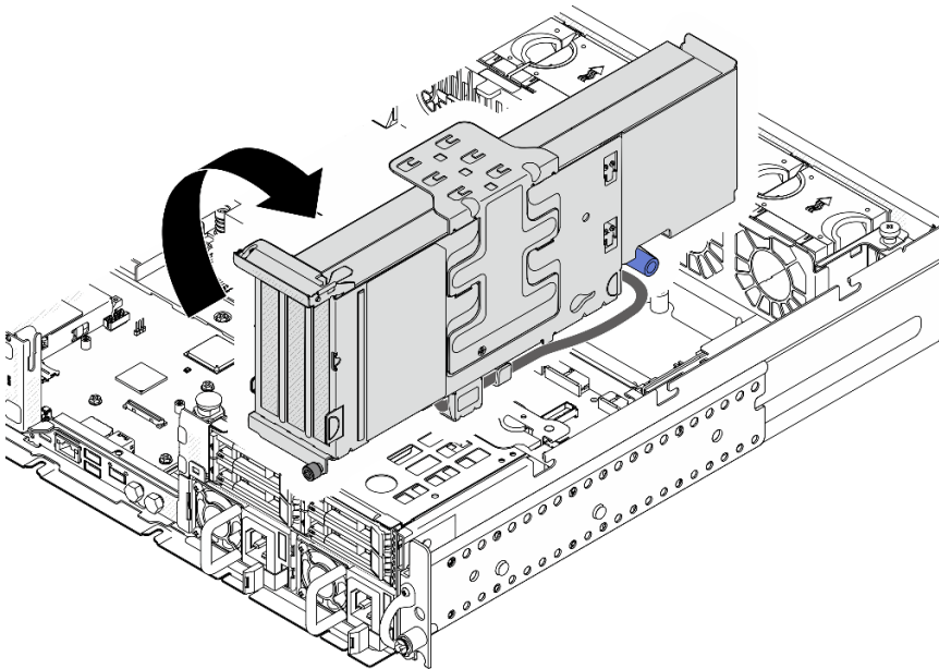
圖例 114. 將 PCIe 擴充卡 2 放在機箱旁邊
