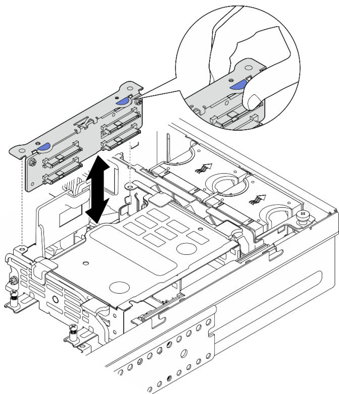
圖例 73. 安裝內部硬碟背板
