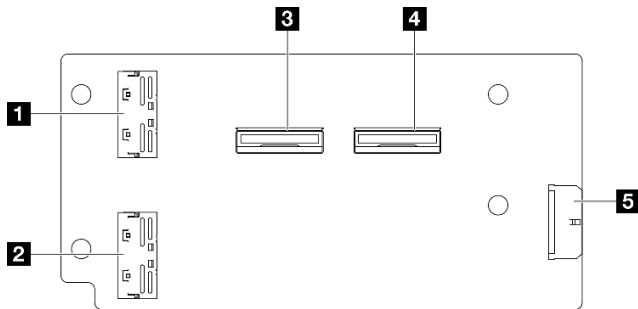
圖例 200. PCIe 擴充卡 2 擴充卡
