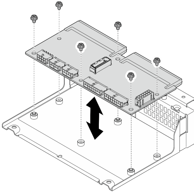
圖例 150. 卸下電源配送板
