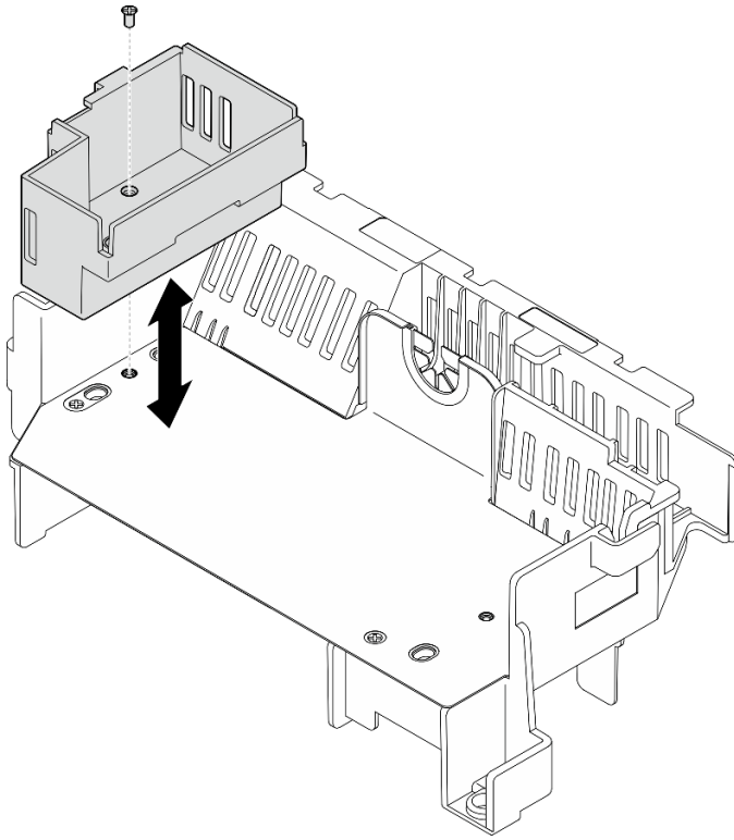
圖例 33. 更換擴充卡 1 填充板
