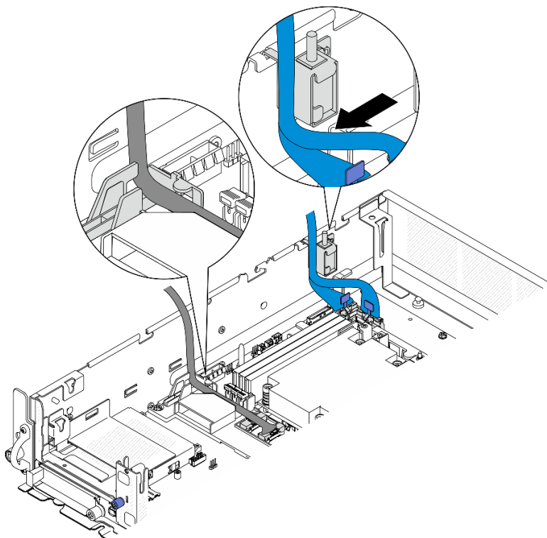
圖例 208. PCIe 擴充卡 1 纜線佈線
