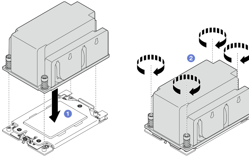
圖例 162. 2U 散熱槽安裝
