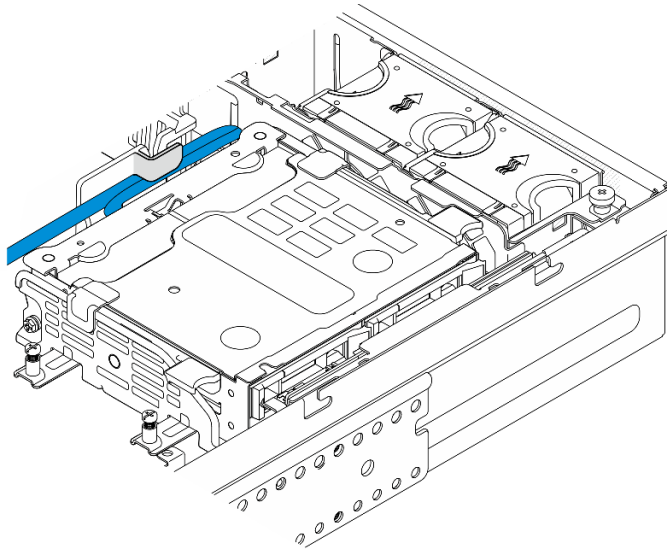
圖例 74. 內部硬碟背板纜線佈線
