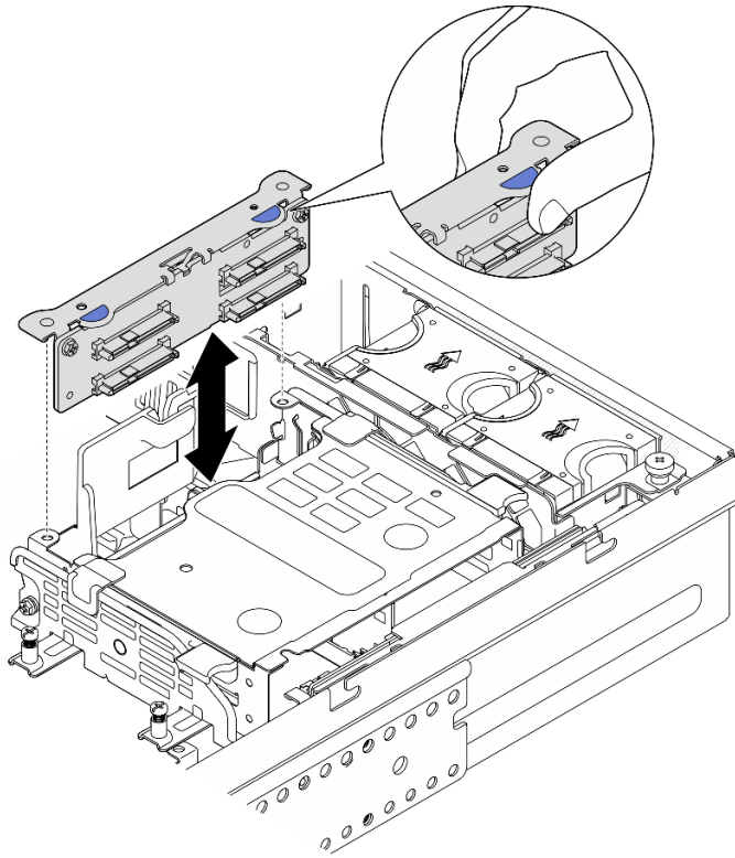
圖例 66. 卸下內部硬碟背板
