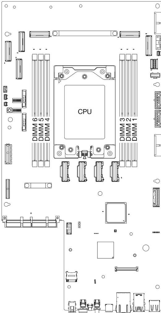
圖例 1. 記憶體模組和處理器佈置
