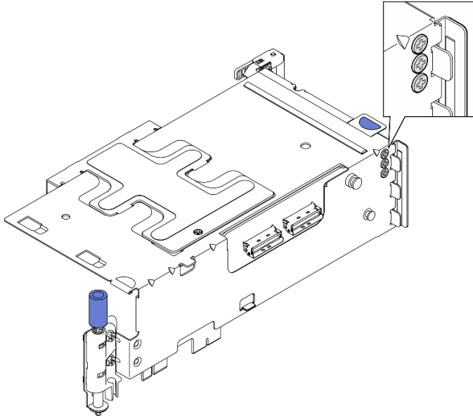
圖例 127. PCIe 擴充卡 1 上的備用螺絲
