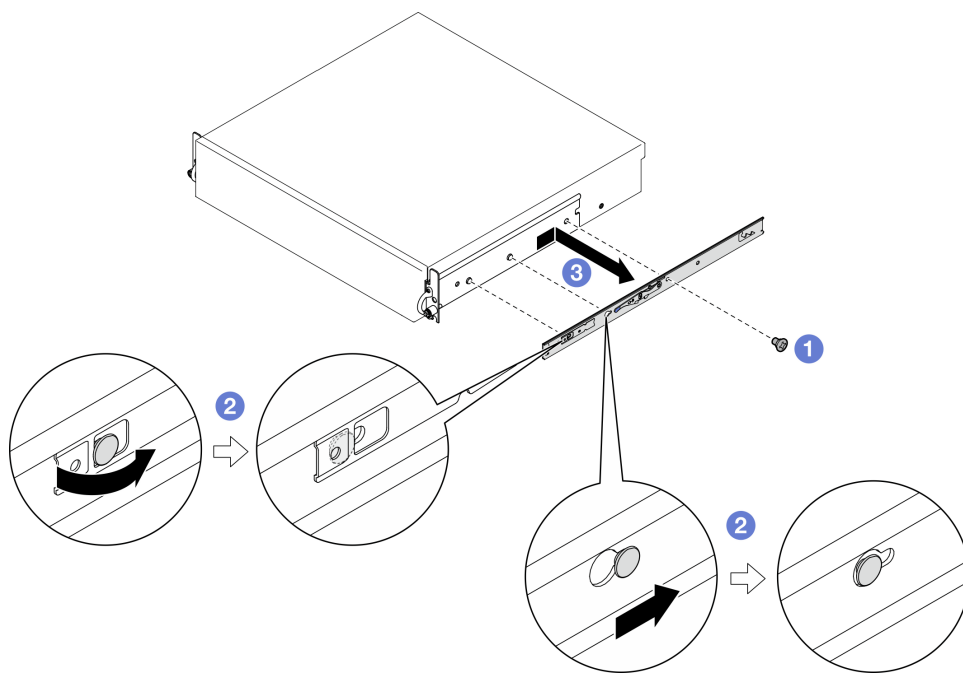
圖例 5. 卸下內滑軌
