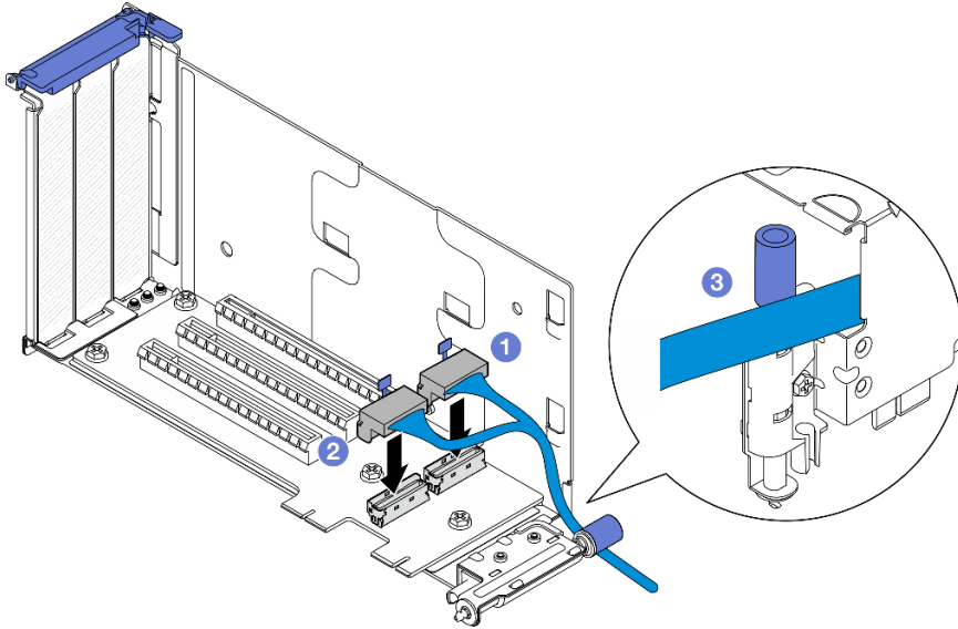
圖例 145. PCIe 擴充卡 1 纜線佈線
