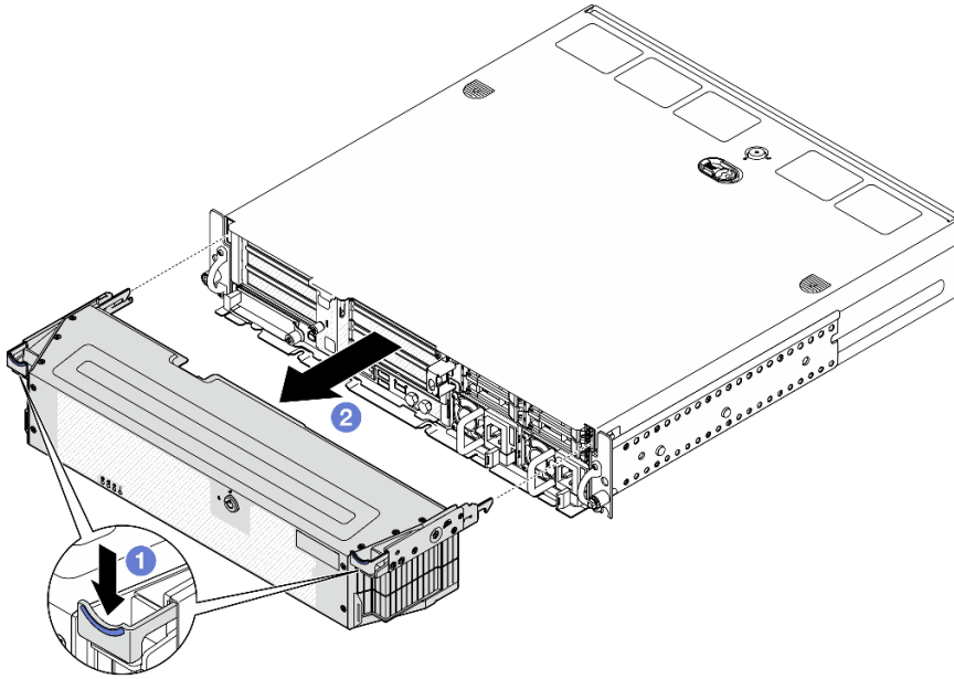
圖例 171. 卸下安全擋板
