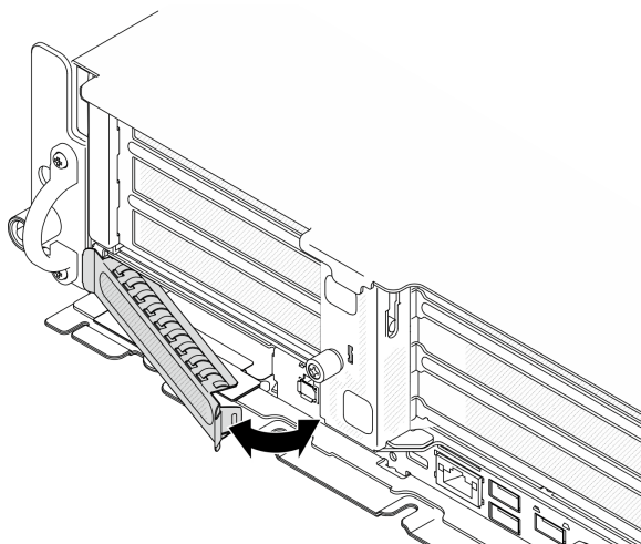
圖例 104. 卸下 OCP 填充板
