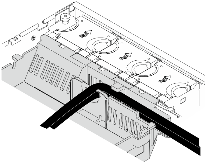
圖例 138. 處理器空氣擋板上的 GPU 電源線
