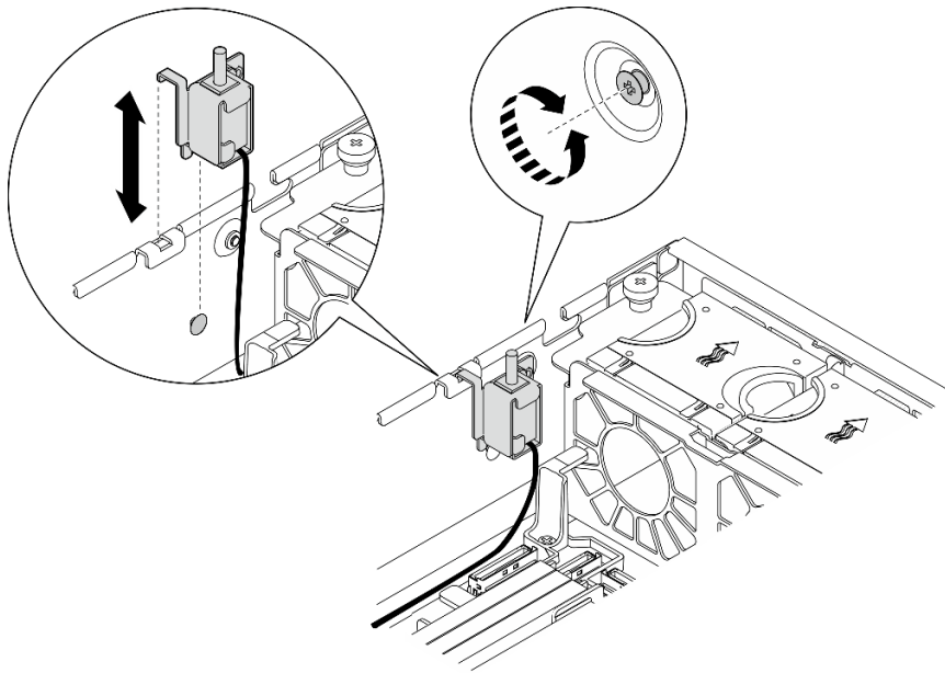
圖例 79. 卸下入侵開關及纜線
