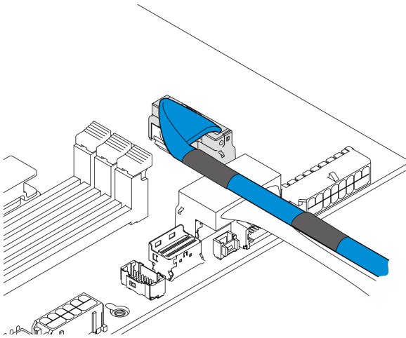
圖例 219. 內部背板信號線
