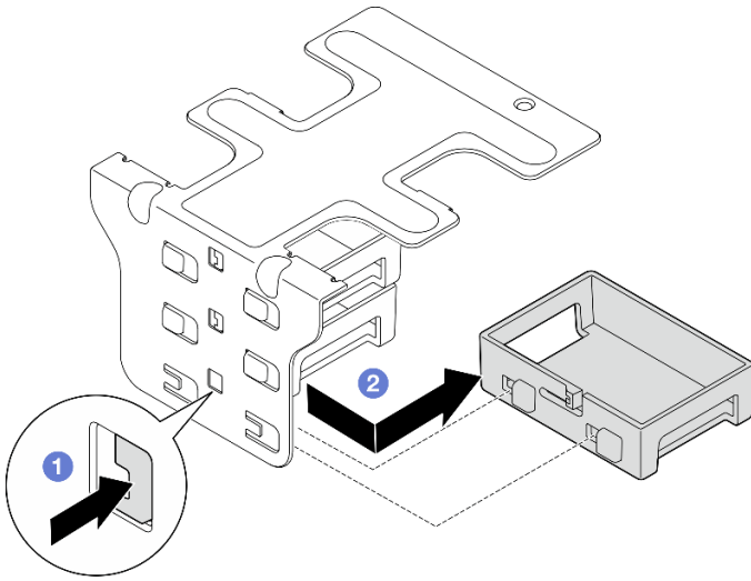
圖例 116. 卸下半高填充板
