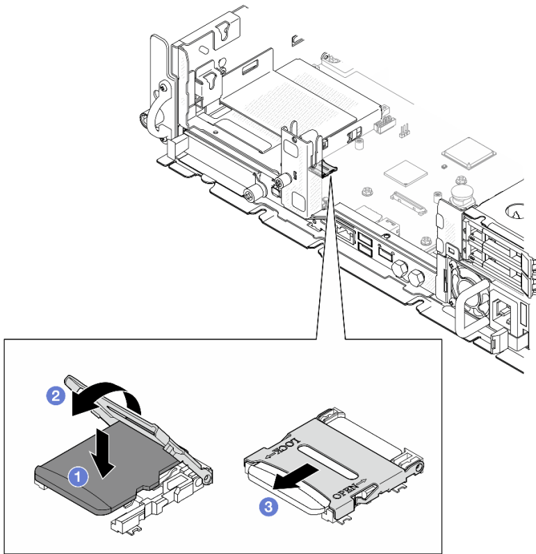
圖例 101. 安裝 MicroSD 卡
