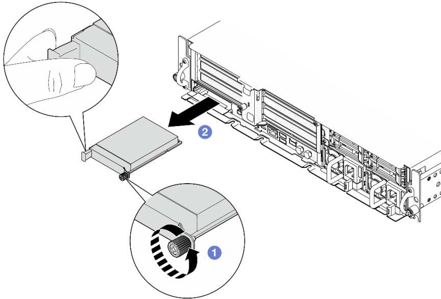
圖例 102. 卸下 OCP 模組
