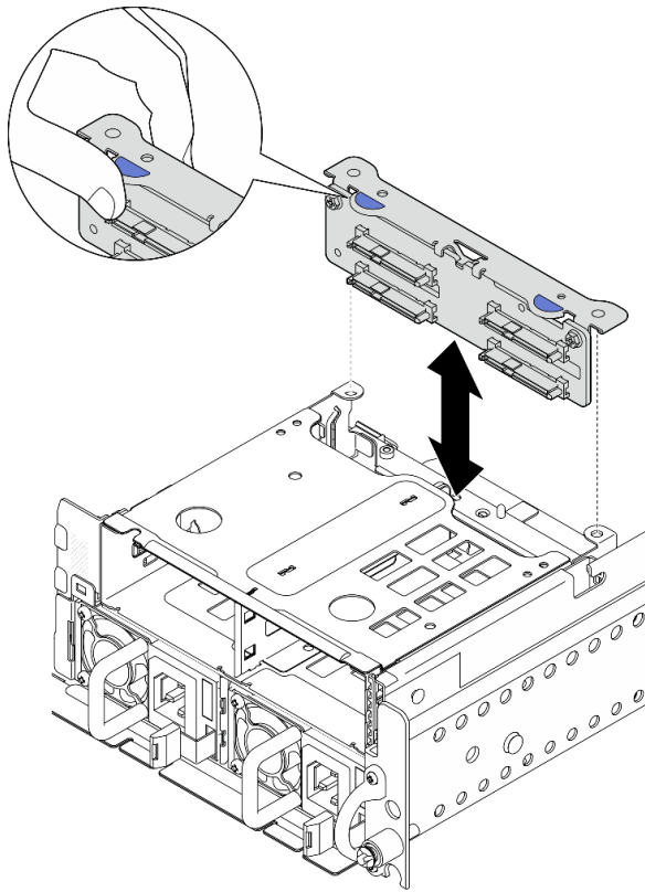
圖例 56. 卸下前方硬碟背板
