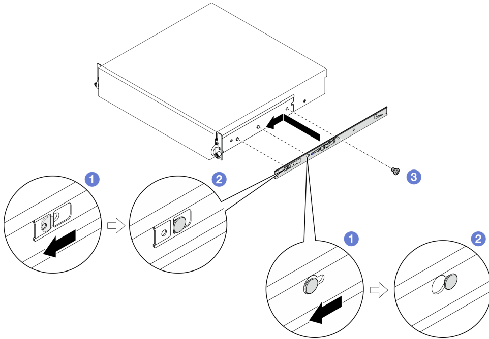
圖例 16. 安裝內滑軌
