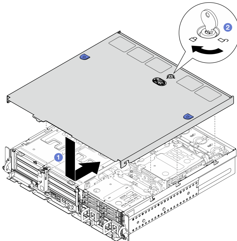
圖例 193. 安裝上蓋
