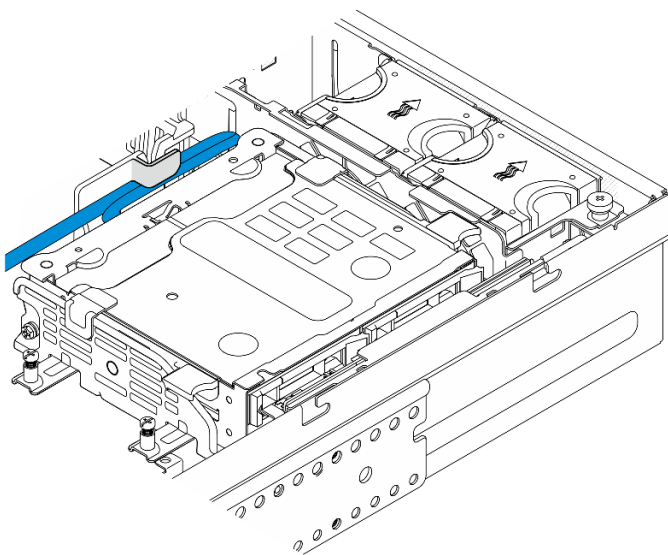
圖例 140. 整理纜線
