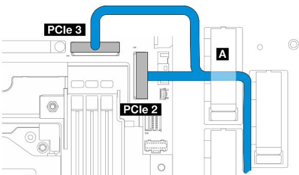
圖例 215. 內部背板信號線
