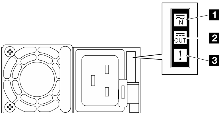
圖例 232. 電源供應器 LED
