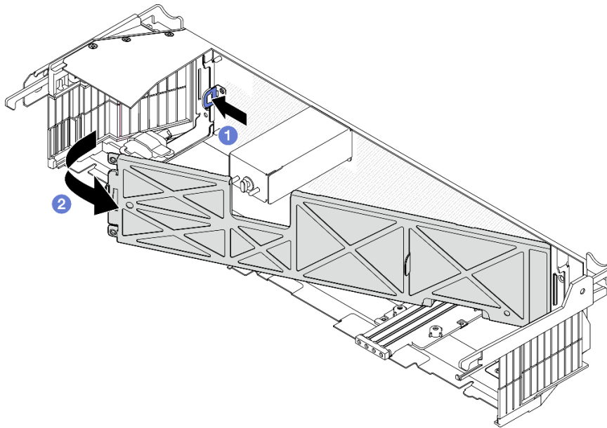
圖例 172. 卸下灰塵過濾器
