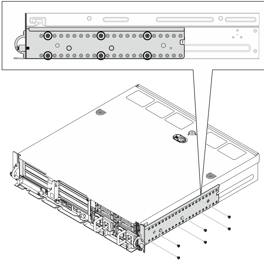
圖例 14. EIA 托架一般深度 1 到 6 : 六顆螺絲
