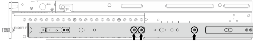
圖例 10. ThinkEdge 1000 公釐摩擦滑軌套件 v2 的內滑軌的三顆螺絲
