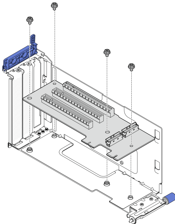
圖例 142. 從 PCIe 擴充卡 1 卸下擴充卡
