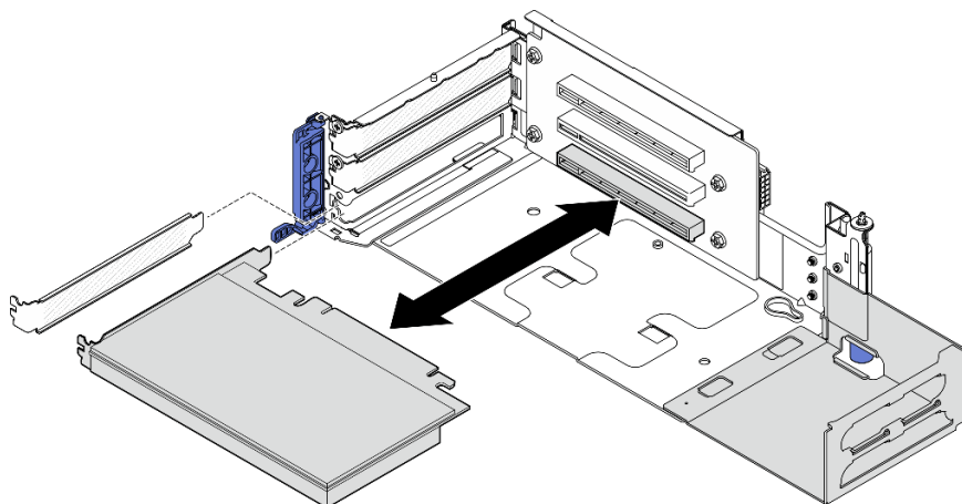
圖例 125. 將 PCIe 配接卡安裝至 PCIe 擴充卡 2
