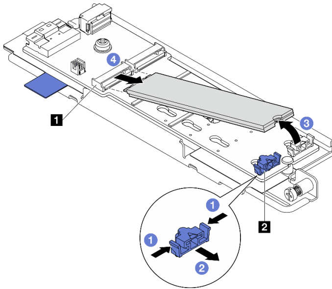
圖例 85. 卸下 M.2 硬碟
