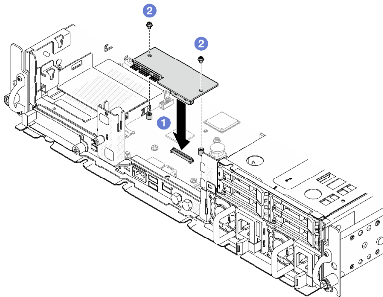
圖例 185. 安裝韌體和 RoT 安全模組
