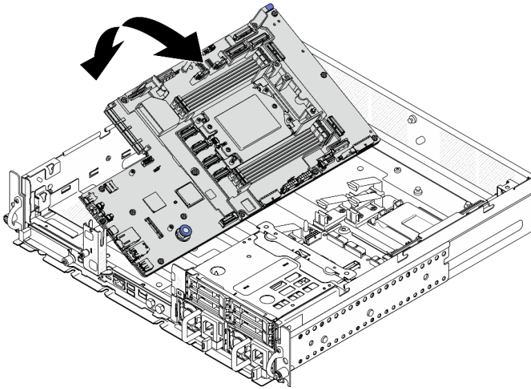
圖例 187. 卸下主機板
