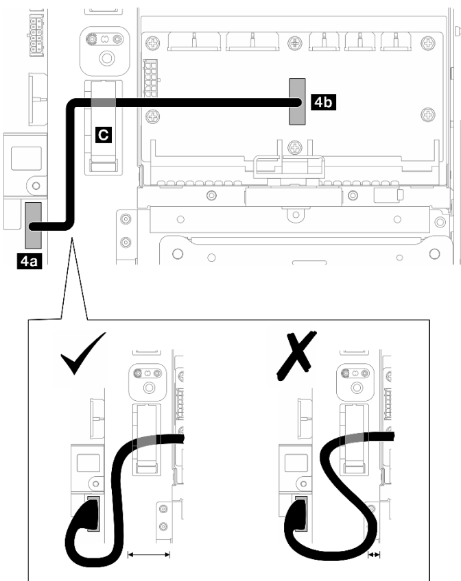
圖例 204. PDB 側頻纜線佈線
