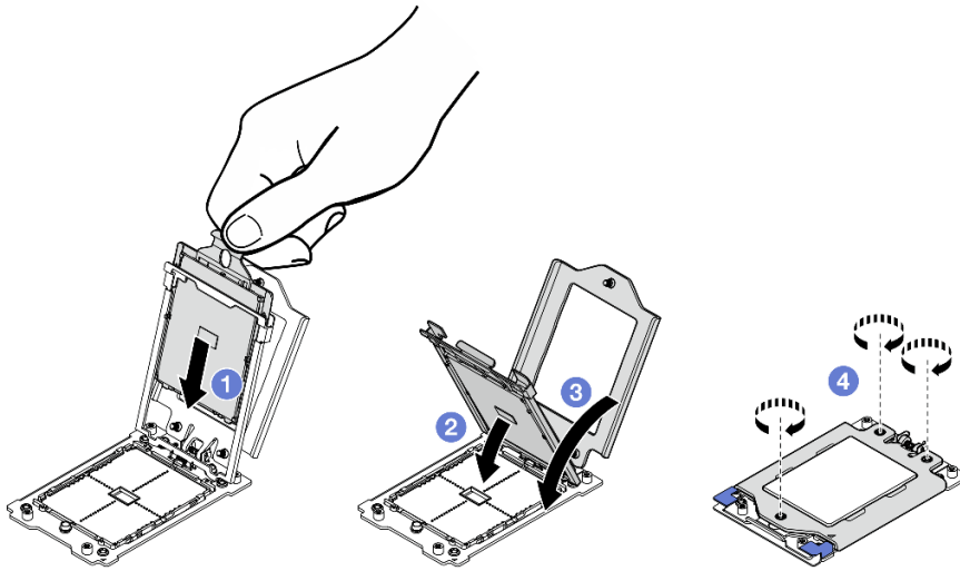
圖例 159. 安裝處理器
