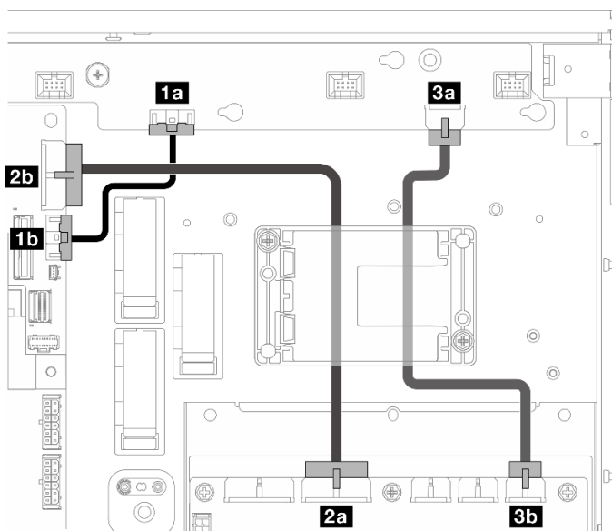
圖例 203. PDB 和 FCB 纜線佈線
