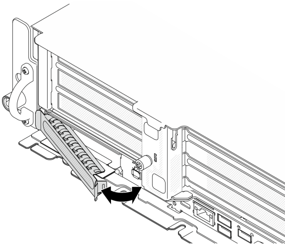
圖例 103. 安裝 OCP 填充板
