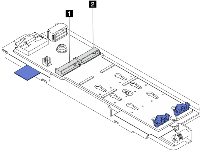
圖例 84. M.2 硬碟插槽編號
