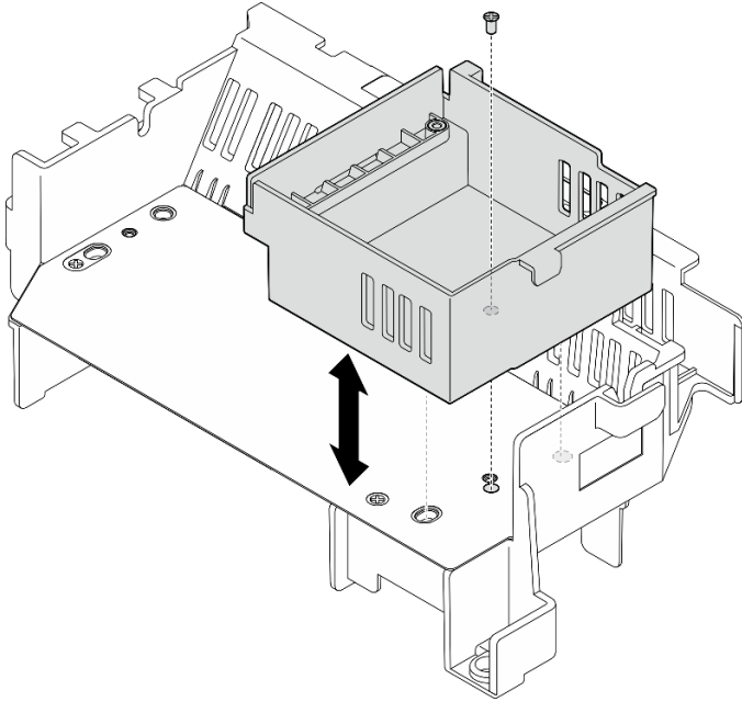
圖例 34. 更換擴充卡 2 填充板
