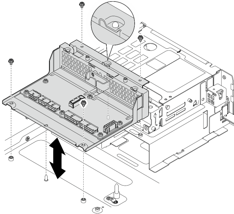
圖例 152. 安裝 PDB 框架
