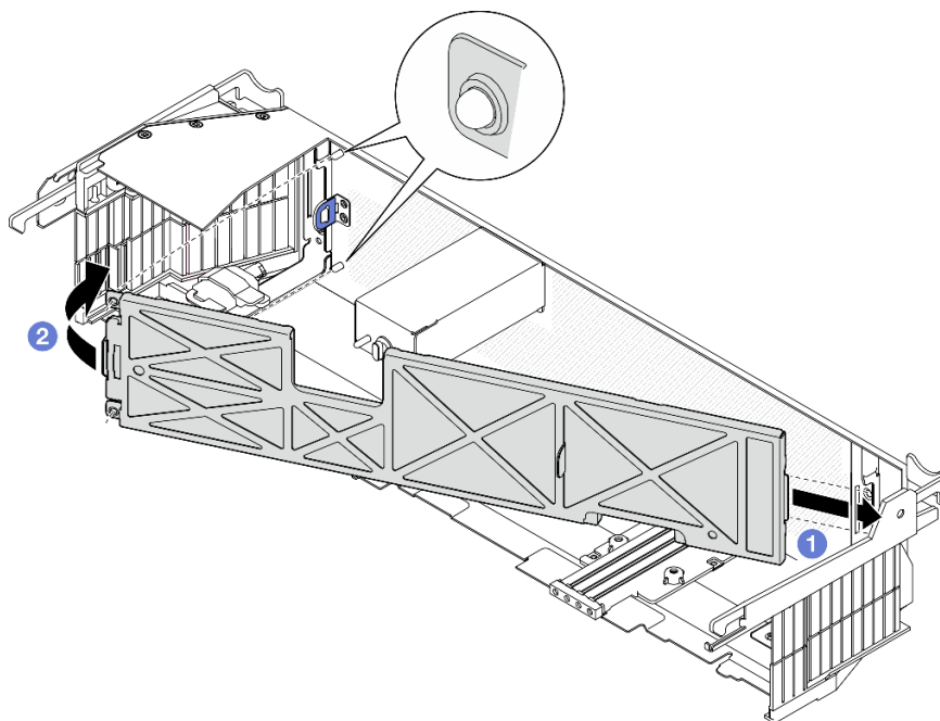
圖例 173. 安裝灰塵過濾器
