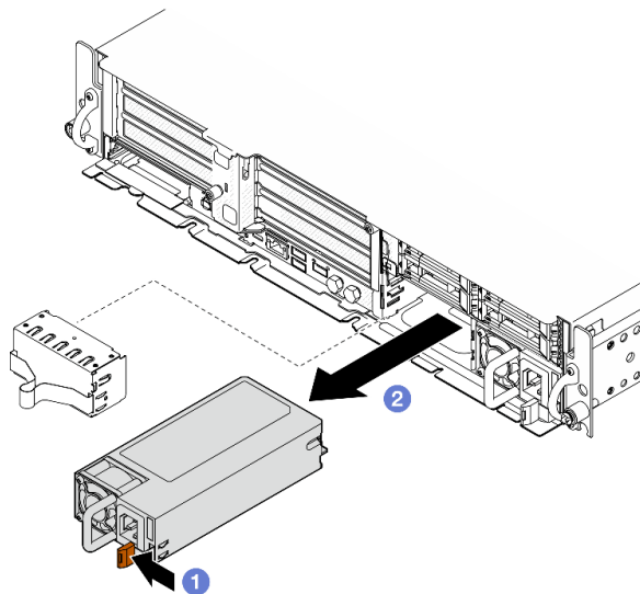
圖例 154. 電源供應器卸下
