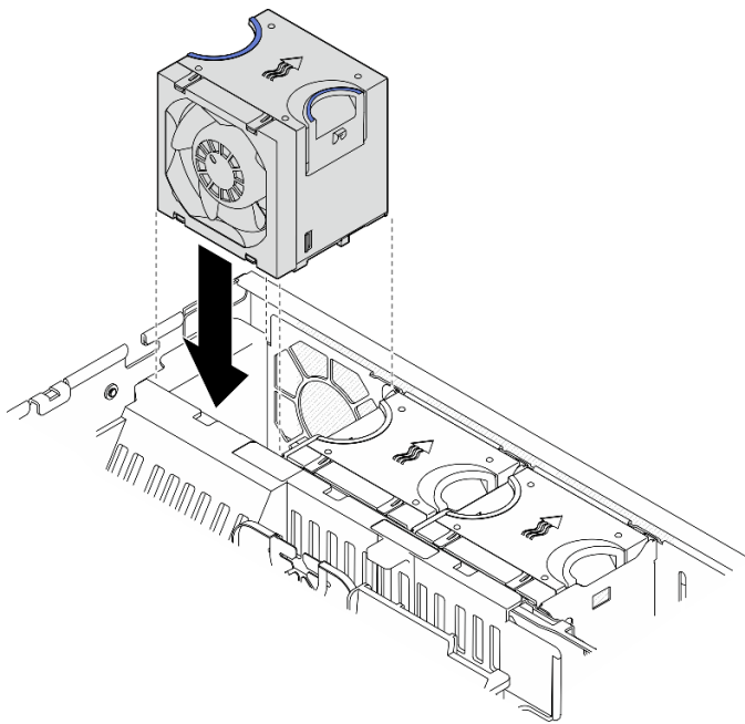
圖例 49. 安裝風扇
