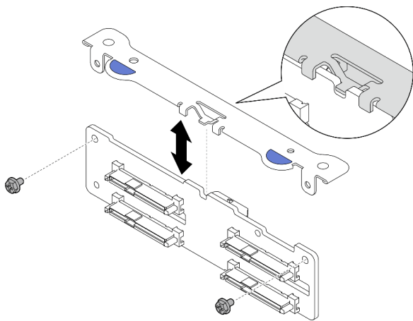
圖例 57. 將硬碟背板與背板托架分開
