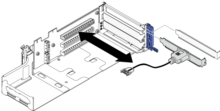
圖例 182. 安裝序列埠模組
