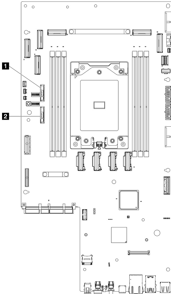
圖例 46. 主機板上的 CMOS 電池位置
