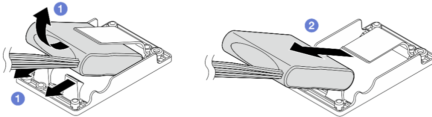
圖例 163. 卸下 RAID 快閃記憶體電源模組
