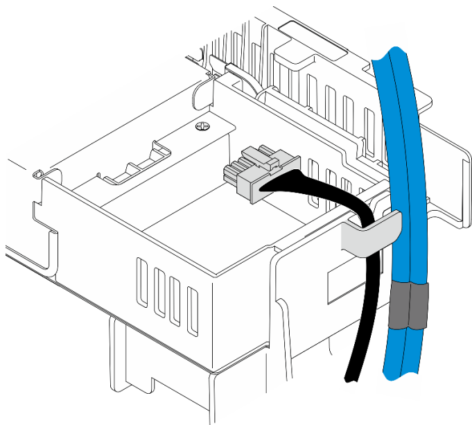
圖例 72. 纜線夾上的內部背板纜線
