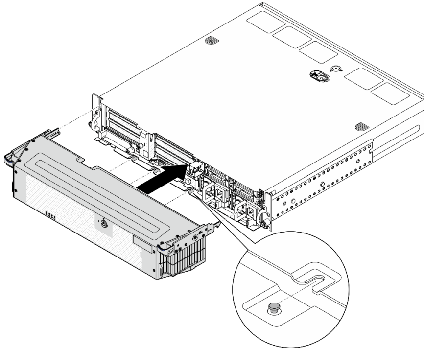
圖例 175. 安裝安全擋板
