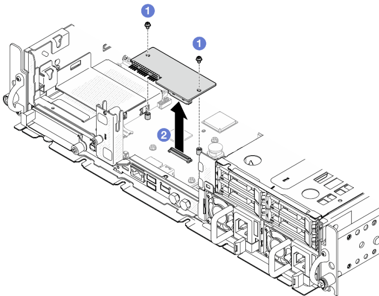
圖例 184. 卸下韌體和 RoT 安全模組
