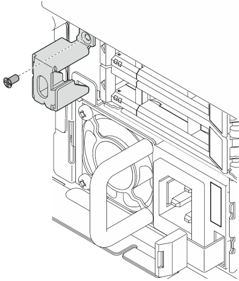
圖例 179. 安裝安全擋板鑰匙鎖托架
