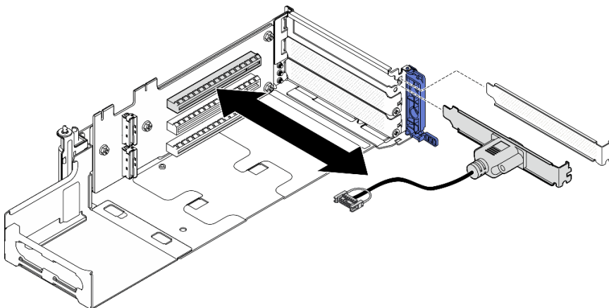
圖例 181. 卸下序列埠模組
