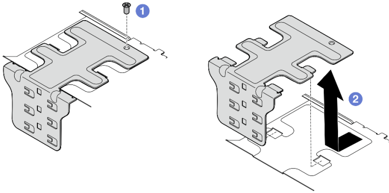
圖例 115. 卸下側面支撐托架
