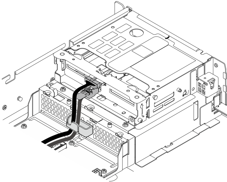
圖例 60. 前方硬碟背板纜線佈線
