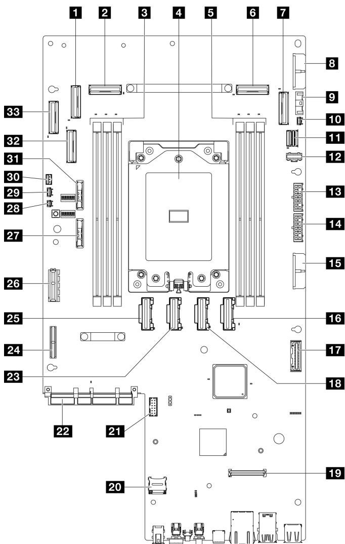
圖例 228. 主機板接頭
