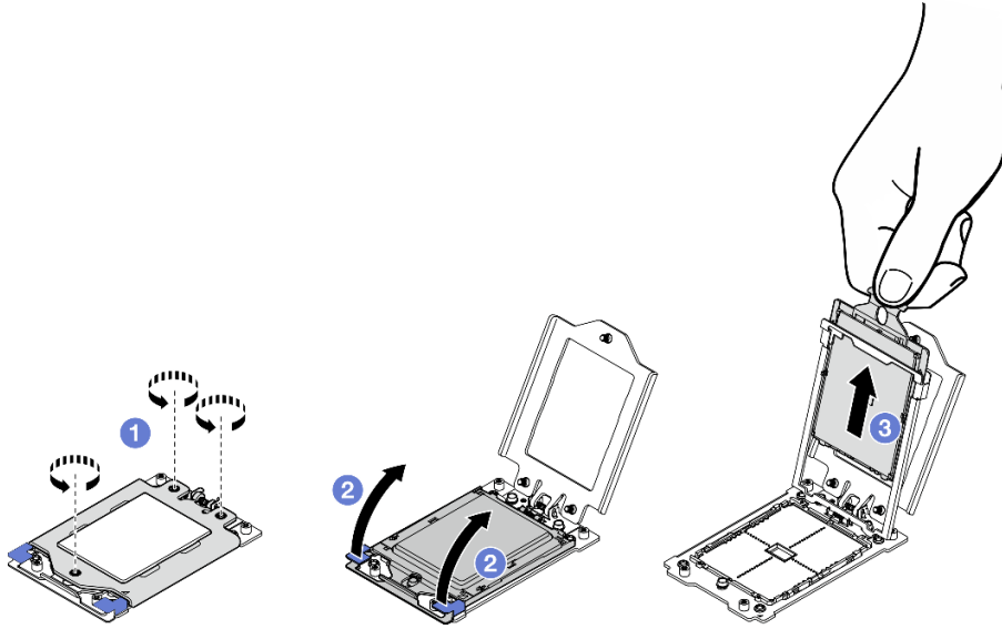
圖例 158. 卸下處理器
