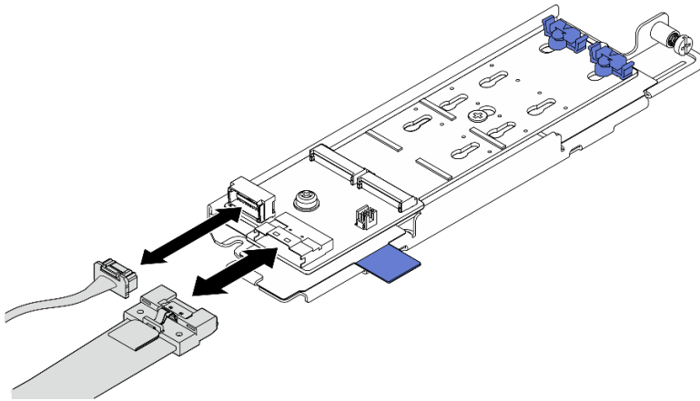
圖例 82. 從 SATA/x4 NVMe M.2 背板拔下纜線
