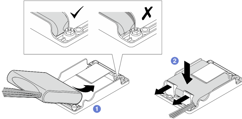
圖例 166. 安裝 RAID 快閃記憶體電源模組
