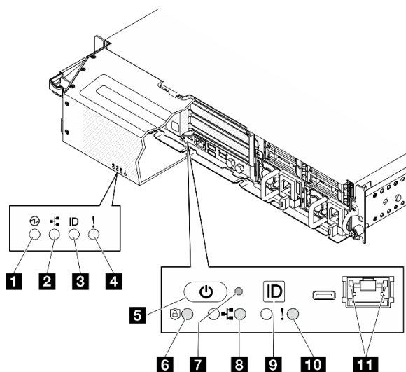
圖例 230. 正面 LED
