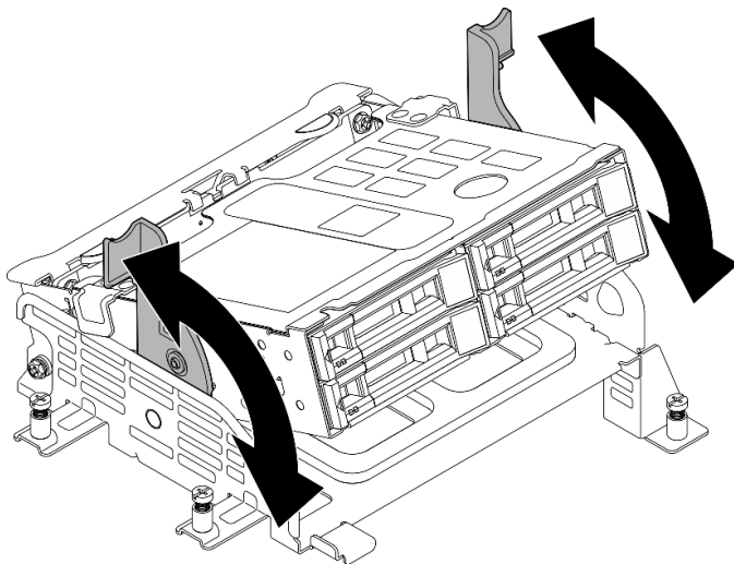
圖例 78. 旋轉內部框架
