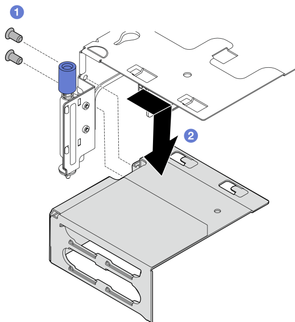
圖例 121. 從 PCIe 擴充卡 2 卸下延伸器
