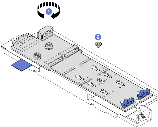
圖例 89. 安裝 M.2 背板
