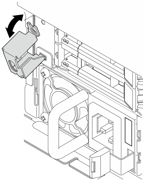
圖例 178. 安裝安全擋板鑰匙鎖托架
