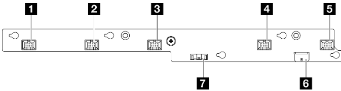
圖例 196. 風扇控制板接頭
