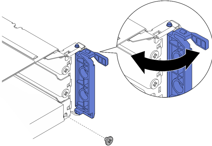
圖例 180. 卸下固定螺絲
