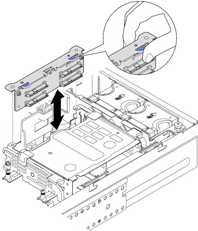
圖例 111. 卸下內部硬碟背板
