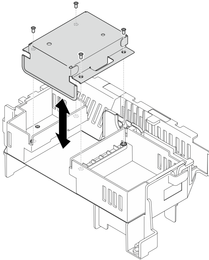
圖例 35. 更換中間填充板
