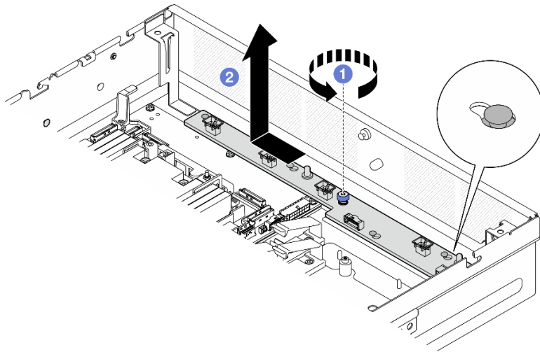
圖例 51. 卸下風扇控制板
