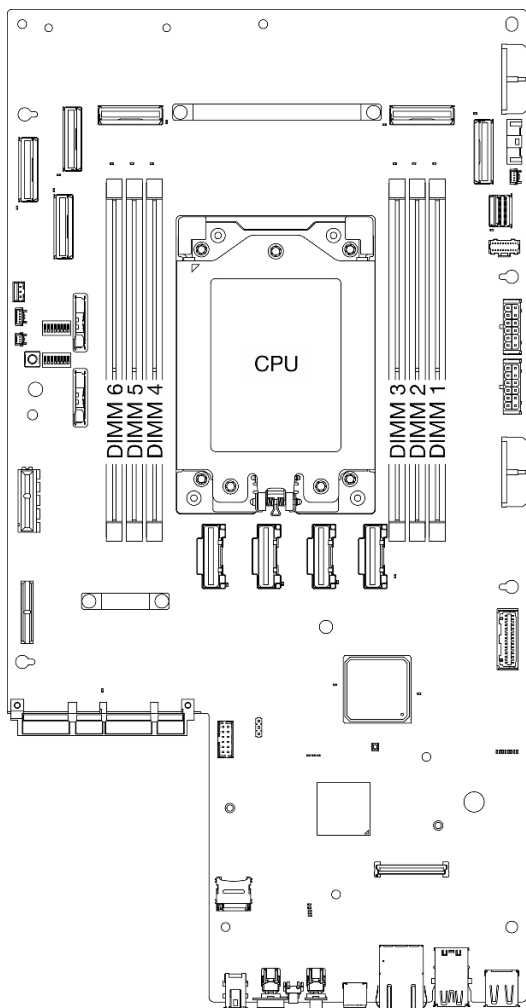
圖例 98. 記憶體模組和處理器佈置
