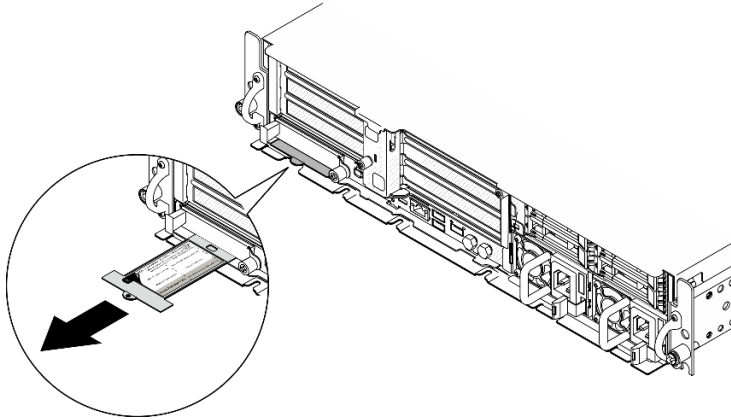
圖例 190. 拉出式資訊標籤上的 Lenovo XClarity Controller 網路存取標籤
