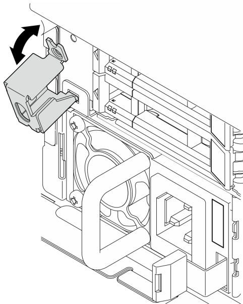
圖例 177. 卸下安全擋板鑰匙鎖托架
