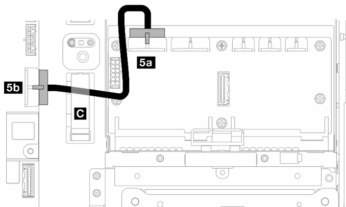
圖例 205. 主機板電源 1 纜線佈線
