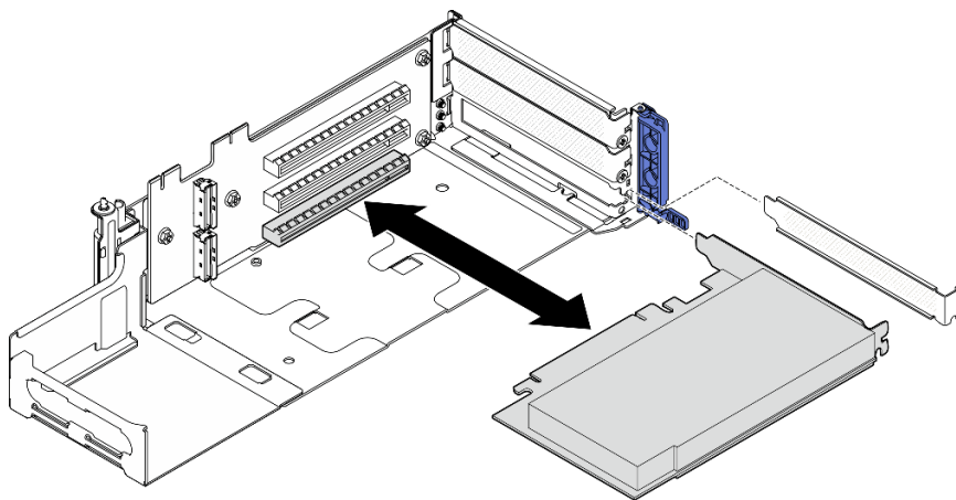
圖例 124. 將 PCIe 配接卡安裝至 PCIe 擴充卡 1
