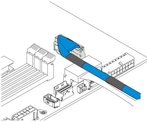
圖例 216. 內部背板信號線
