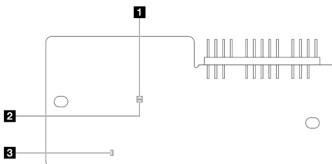
圖例 234. 韌體和 RoT 安全模組上的 LED
