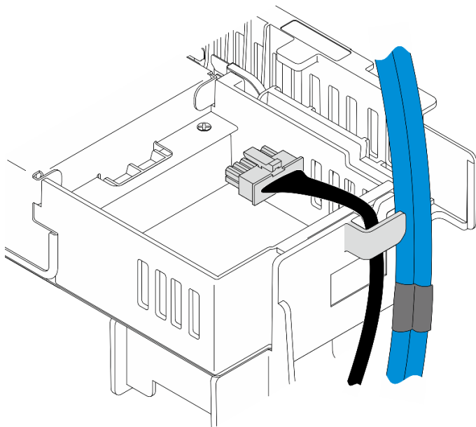
圖例 69. 纜線夾上的內部背板纜線
