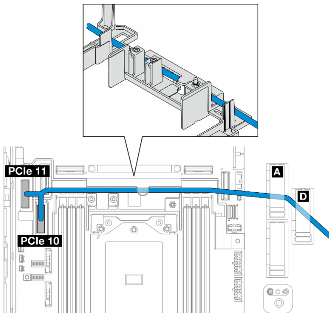
圖例 217. 前方背板信號線
