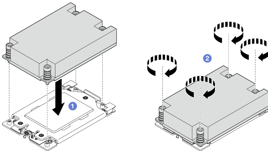
圖例 161. 1U 散熱槽安裝
