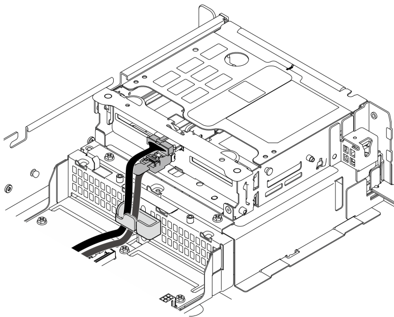
圖例 224. 前方硬碟背板纜線佈線
