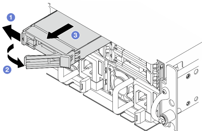
圖例 54. 卸下正面熱抽換硬碟
