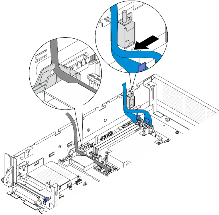
圖例 131. PCIe 擴充卡 1 纜線佈線
