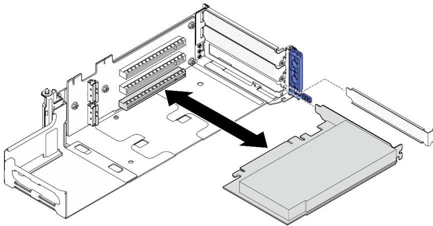
圖例 118. 從 PCIe 擴充卡 1 卸下 PCIe 配接卡
