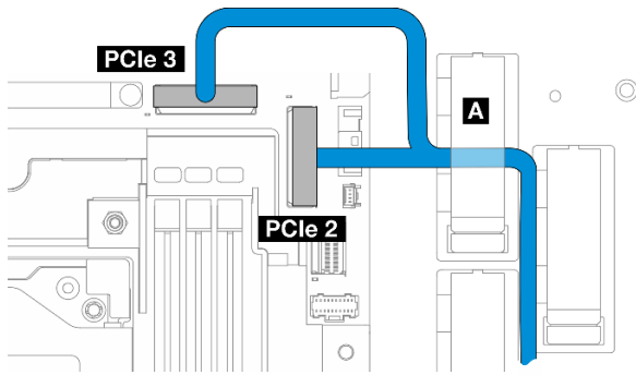
圖例 218. 內部背板信號線
