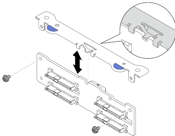
圖例 67. 將硬碟背板與背板托架分開
