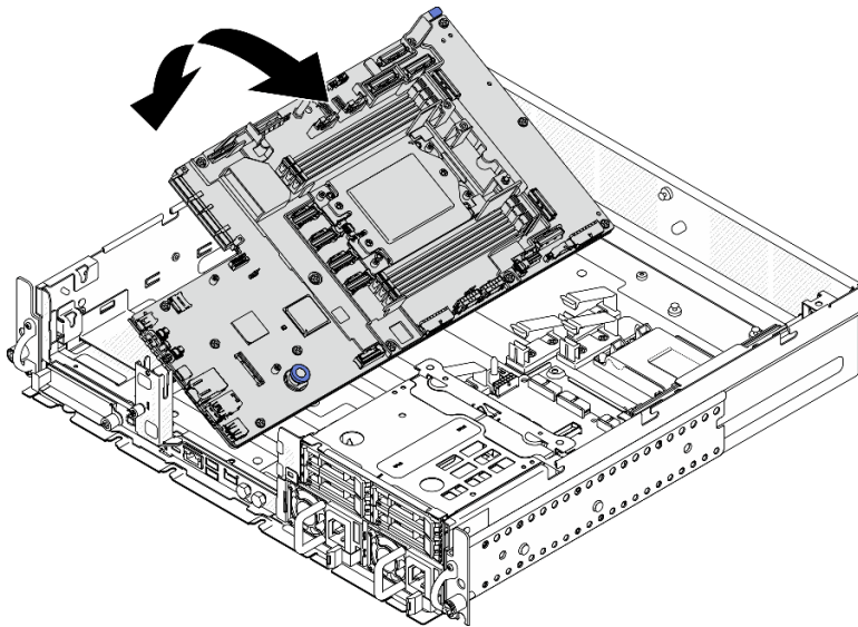
圖例 188. 安裝主機板
