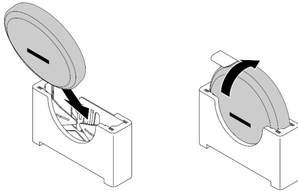
圖例 47. 安裝 CMOS 電池
