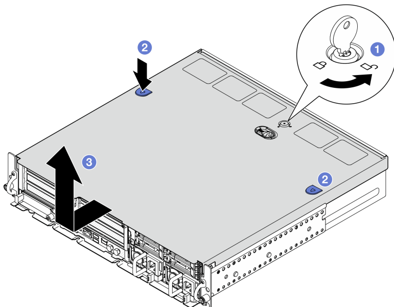
圖例 192. 卸下上蓋
