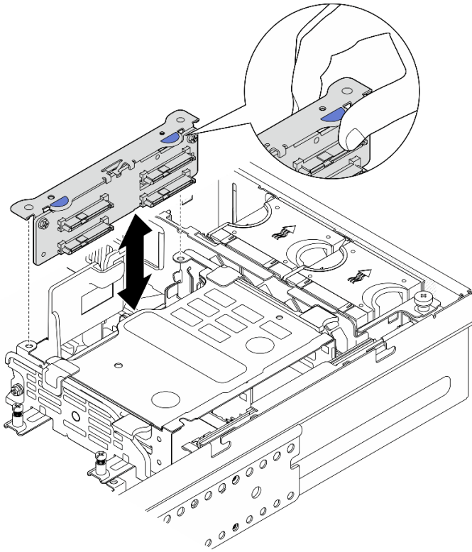
圖例 139. 安裝內部硬碟背板
