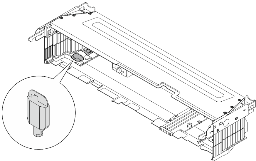
圖例 174. 安全擋板鑰匙存放位置
