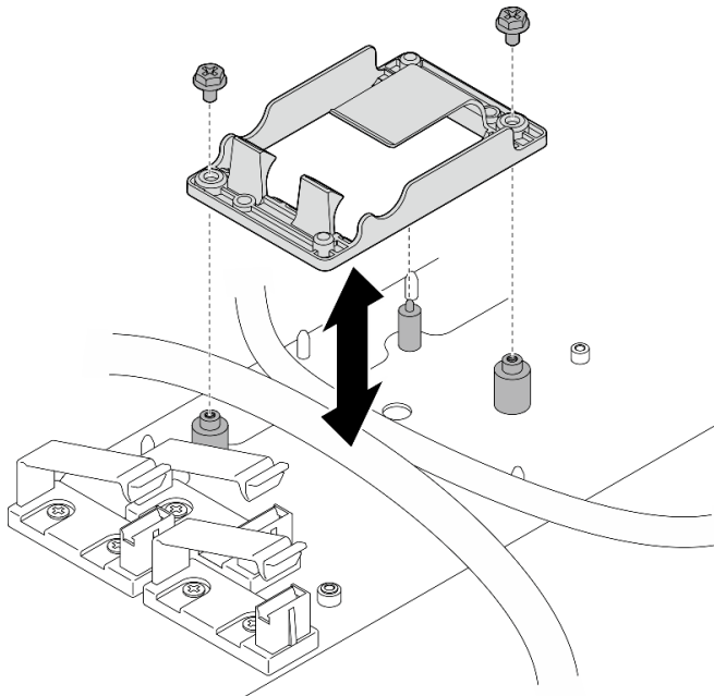
圖例 168. 卸下 RAID 快閃記憶體電源模組匣
