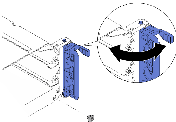
圖例 126. 安裝固定螺絲
