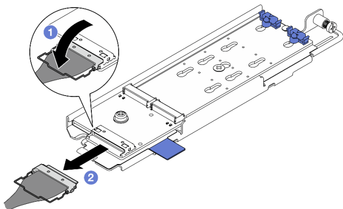
圖例 83. 從 SATA/NVMe M.2 背板拔下纜線
