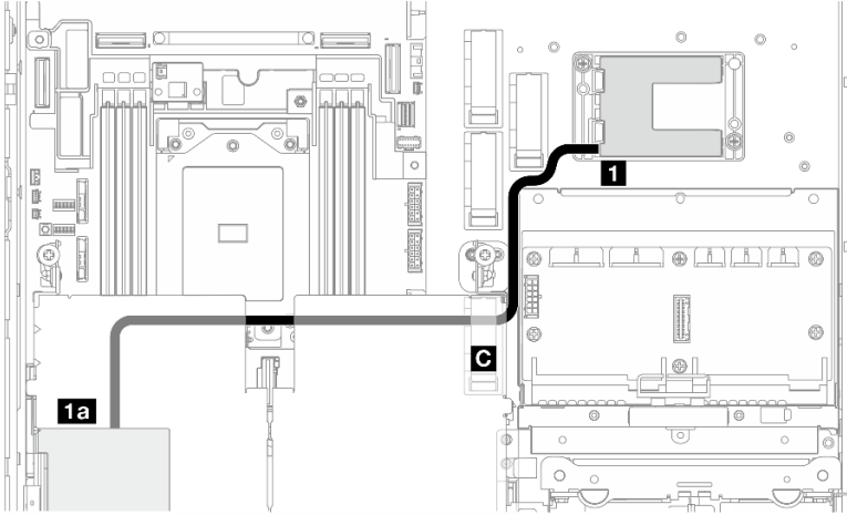
圖例 211. PCIe 擴充卡 1 上的 RAID 配接卡
