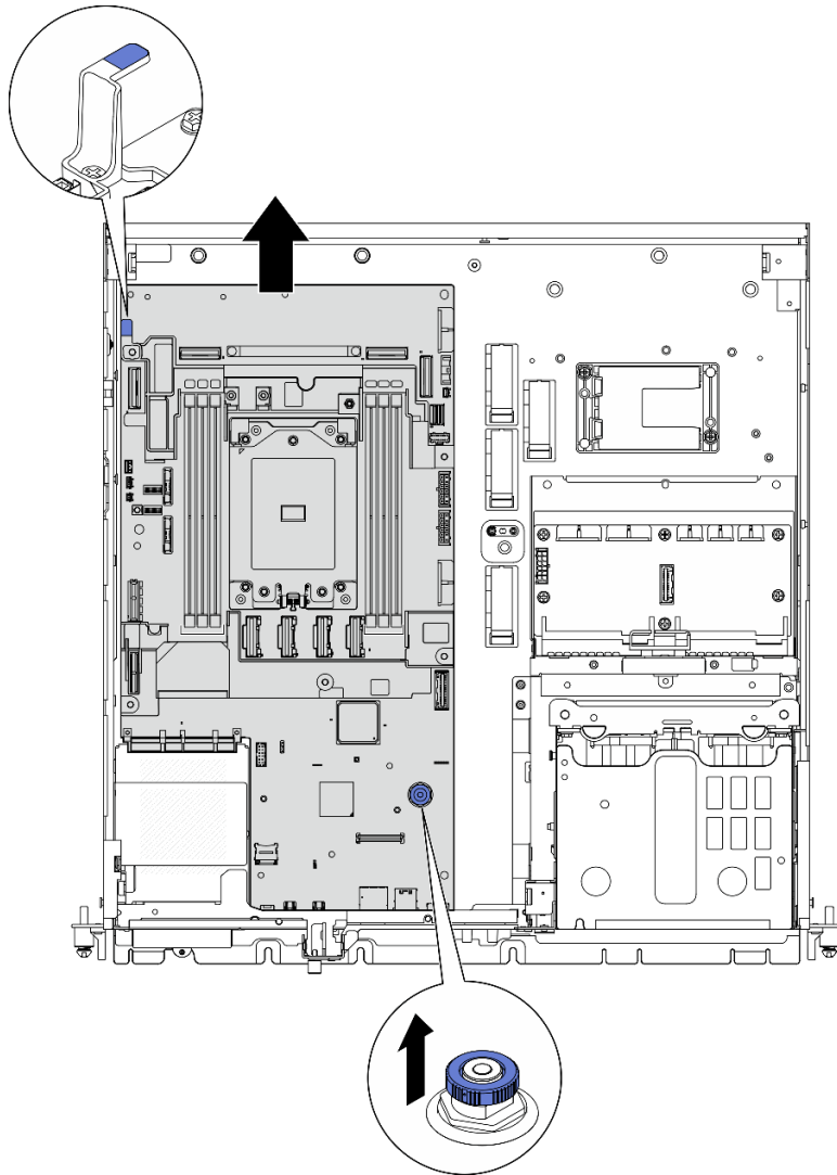
圖例 186. 鬆開主機板
