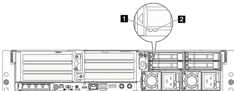
圖例 229. 硬碟 LED
