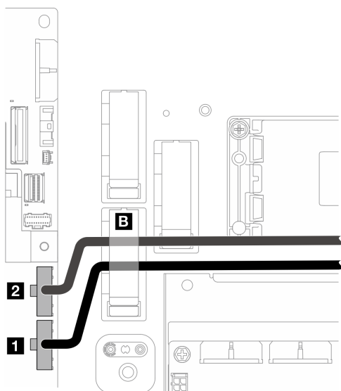
圖例 213. 背板電源線
