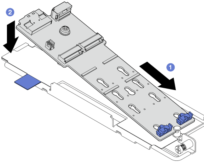
圖例 88. 安裝 M.2 背板
