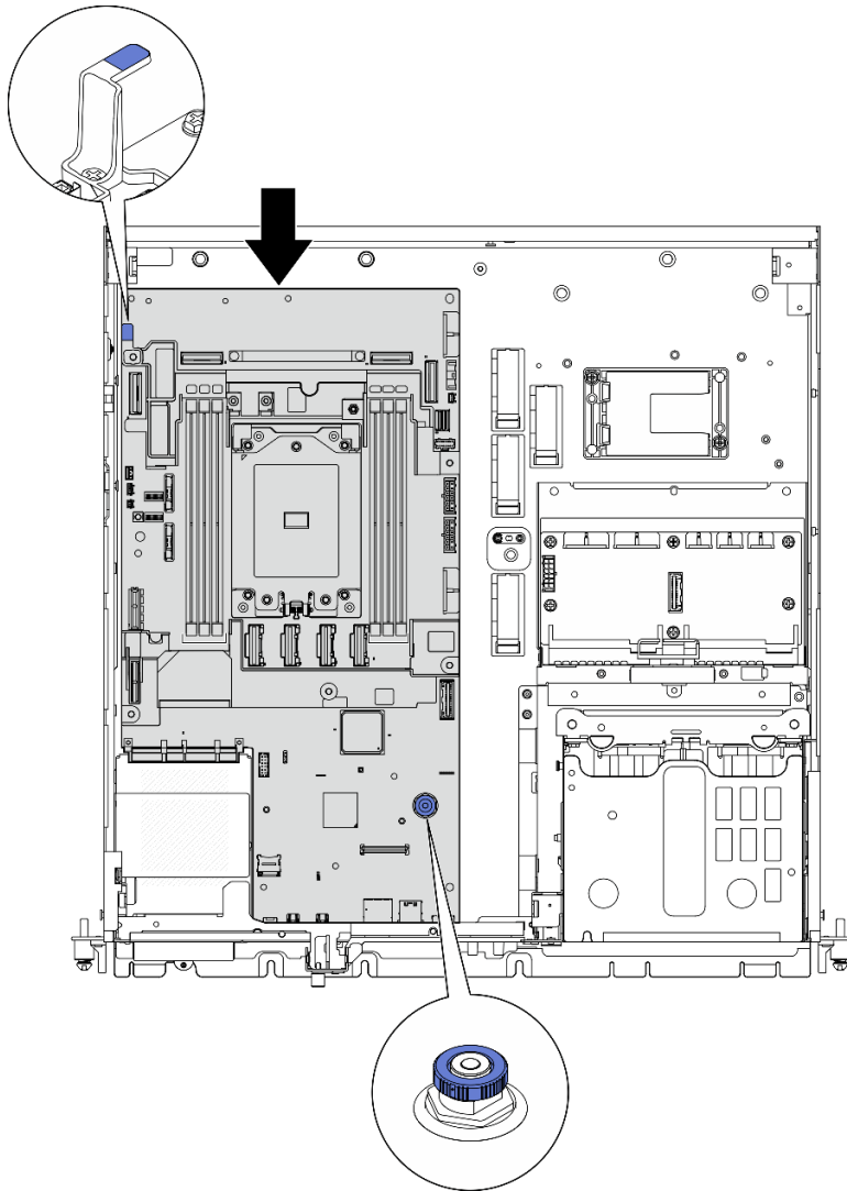
圖例 189. 固定主機板
