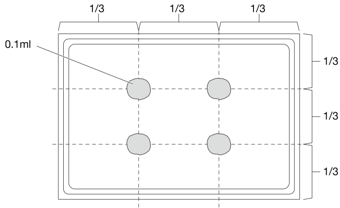
圖例 160. 塗上散熱膏
