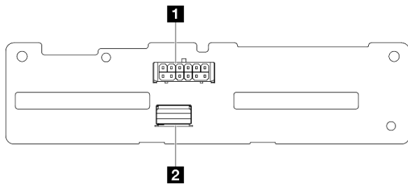
圖例 194. SAS/SATA 背板接頭
