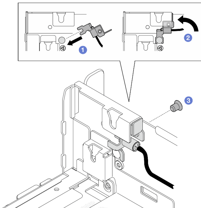
圖例 41. 安裝擋板偵測開關
