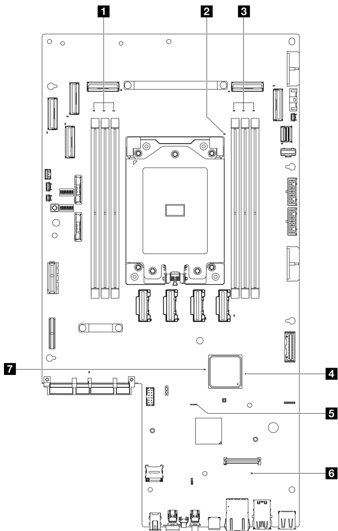
圖例 233. 主機板 LED
