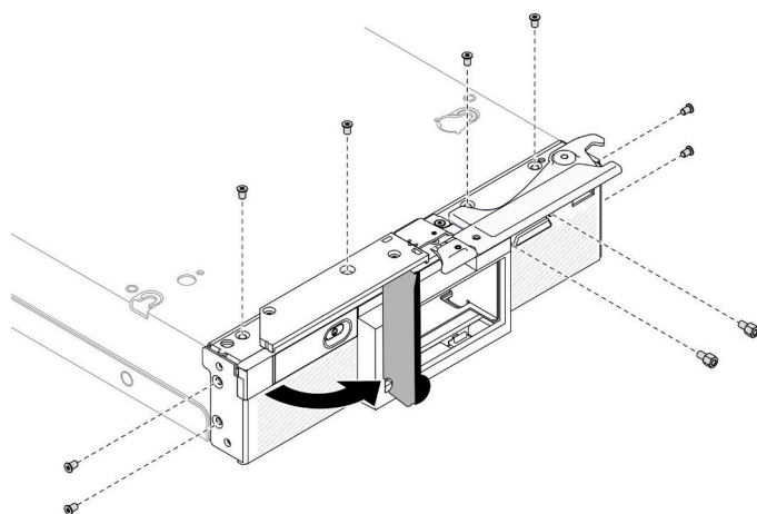
図 78. 前面パネルのねじを緩める
