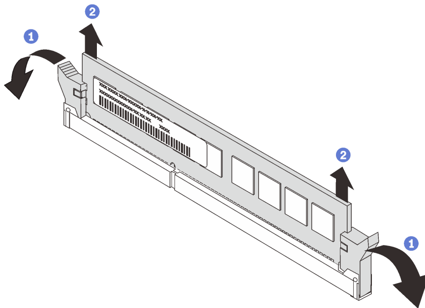
図 46. メモリー・モジュールの取り外し
