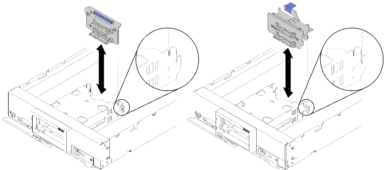
図 13. 2.5 型ドライブ・バックプレーンの取り付け
