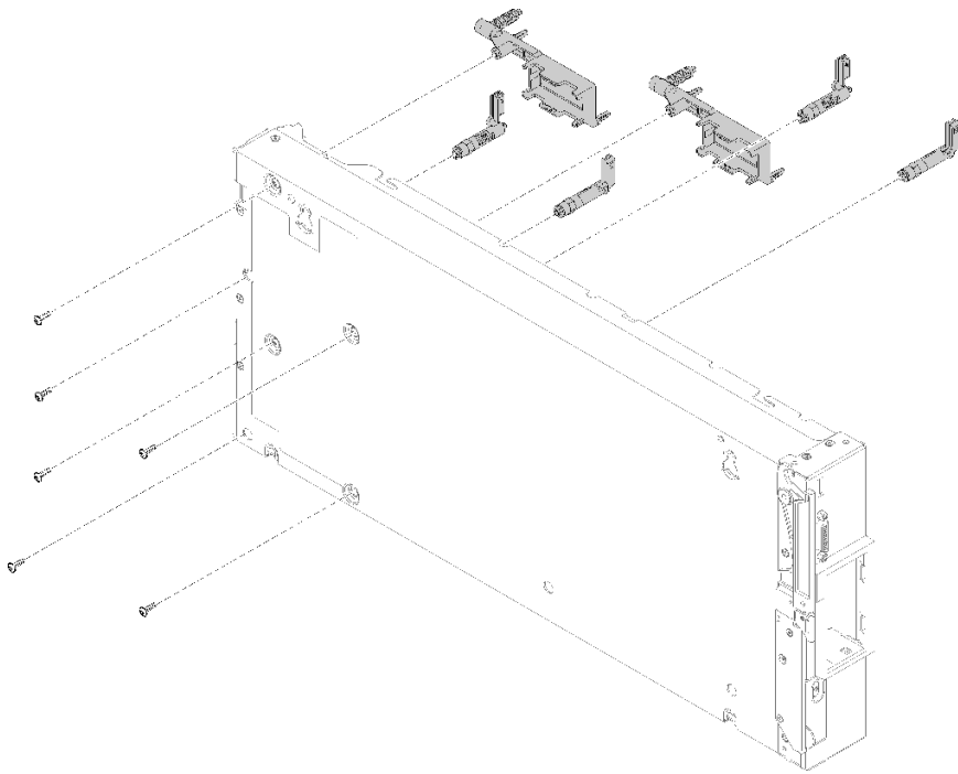
図 17. アダプター保持アセンブリーの取り付け
