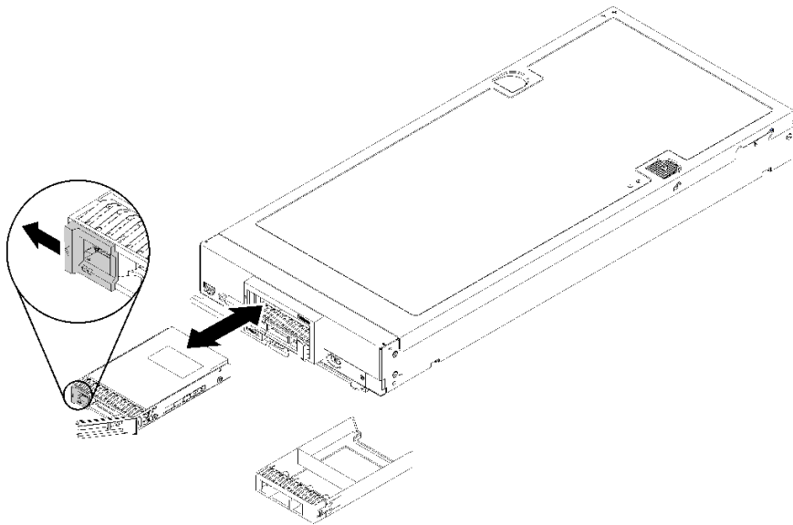
図 10. 2.5 型ホット・スワップ・ドライブの取り外し
