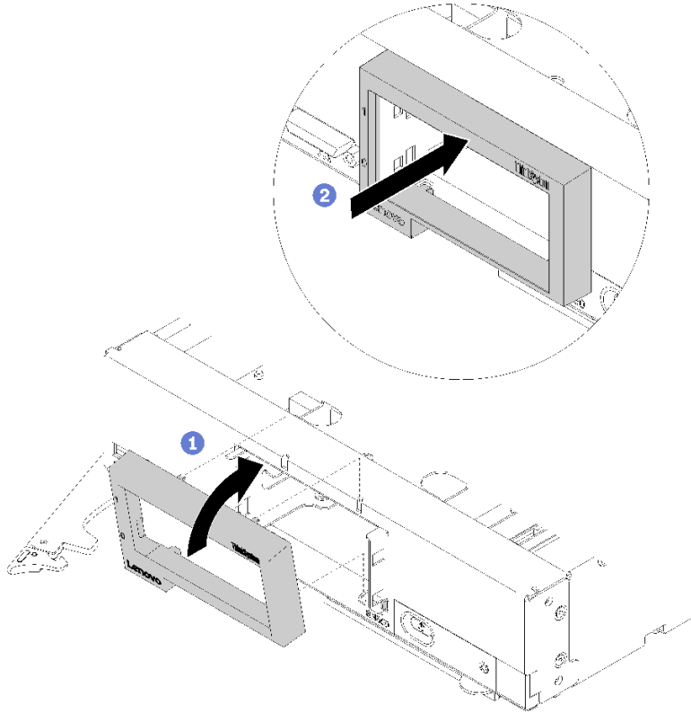
図 19. ベゼルの取り付け
