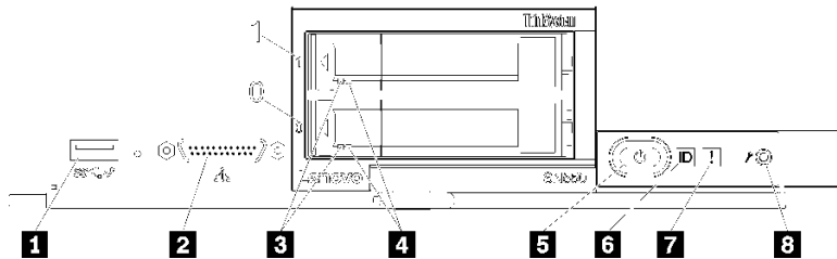
図 73. 計算ノードのコントロール・パネルのボタン、コネクタ、および LED
