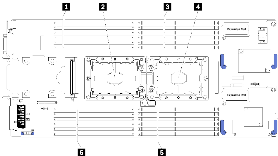
図 57. DIMM とプロセッサの位置
