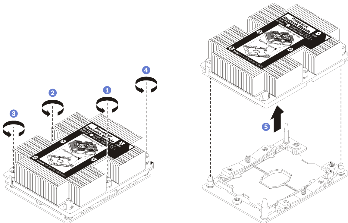
図 51. PHM の取り外し
