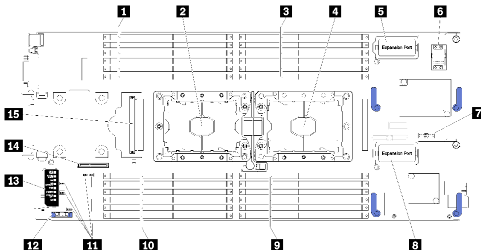
図4. システム・ボード・コネクタ
