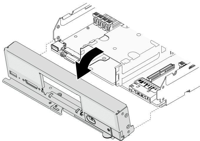
図 79. 前面パネルの取り外し
