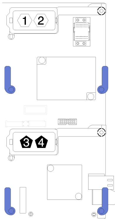
図 36. I/O 拡張コネクタ上の六角形および五角形の番号の位置
