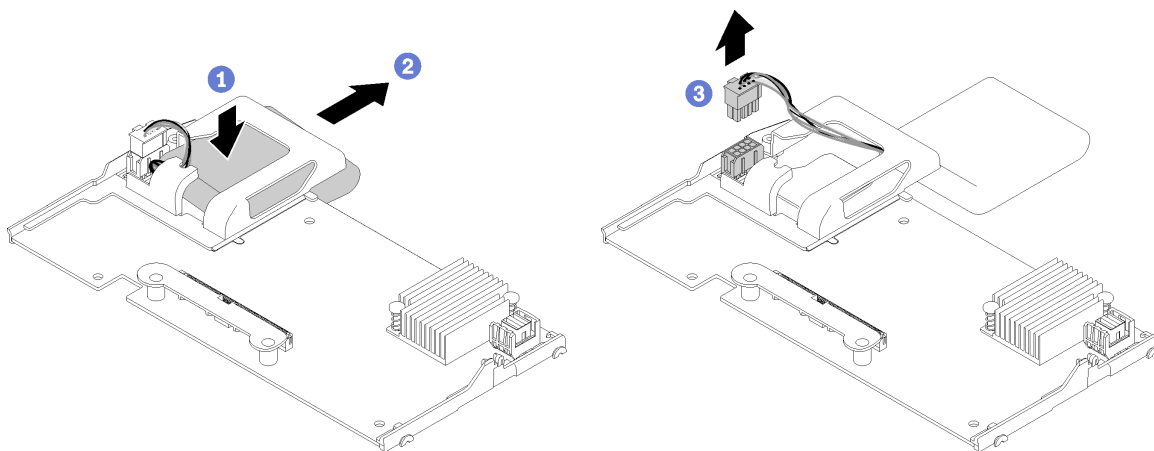
図 28. フラッシュ電源モジュールの取り外し
