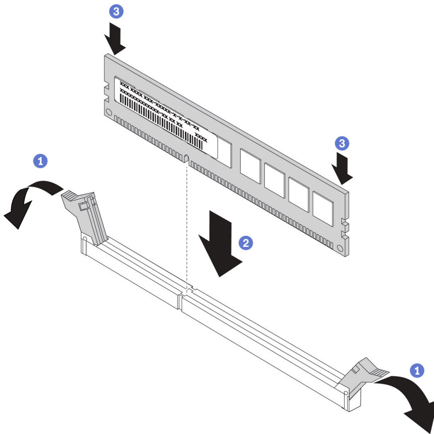
図49. メモリー・モジュールの取り付け
