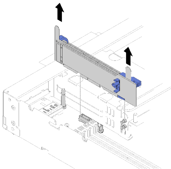
図 38. M.2 バックプレーンの取り外し
