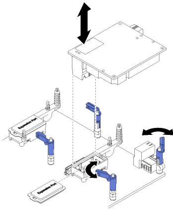
図 37. I/O 拡張アダプターの取り付け
