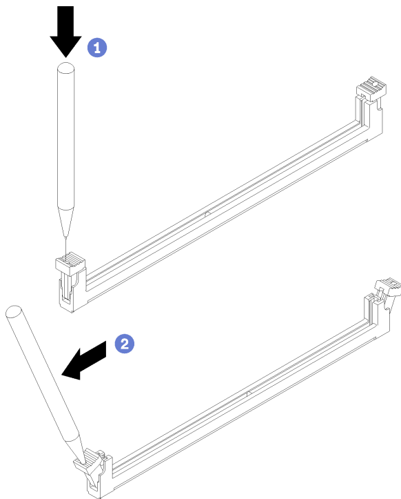
図48. 保持クリップを開く
