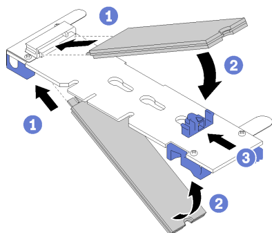
図 43. M.2 ドライブの取り付け
