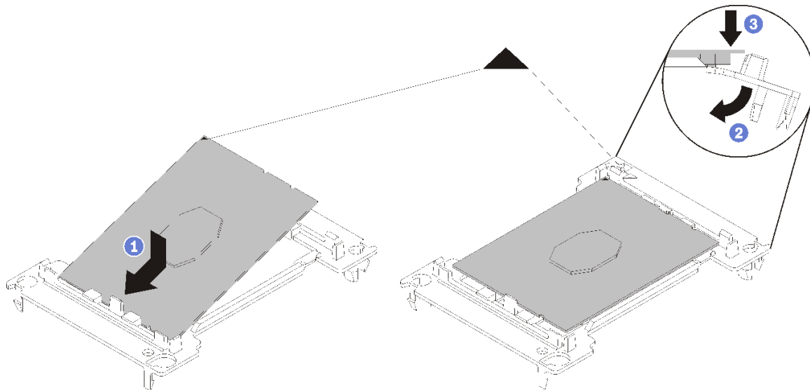
図54. プロセッサ保持器具の取り付け
