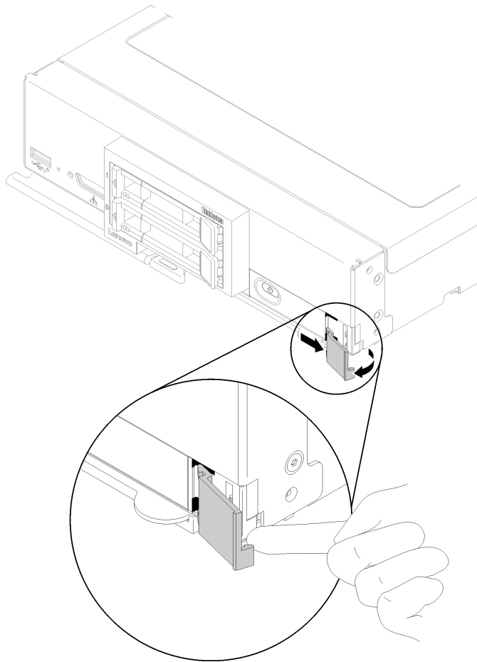
図 32. ID ラベル・プレートの取り外し
