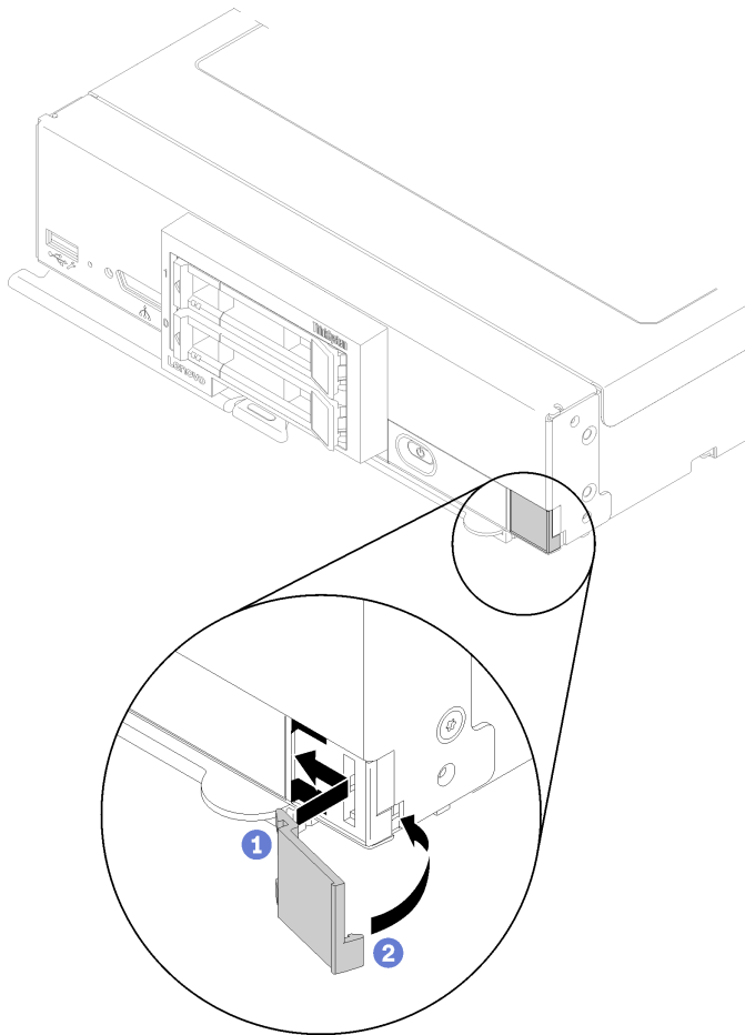
図 33. ID ラベル・プレートの取り付け
