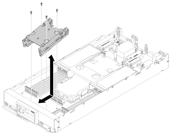
図 65. ストレージ・ケースの取り外し
