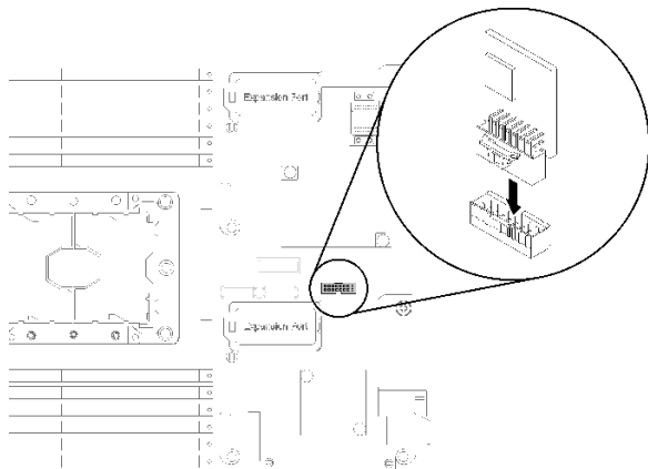
図 69. TCM/TPM アダプターの取り付け
