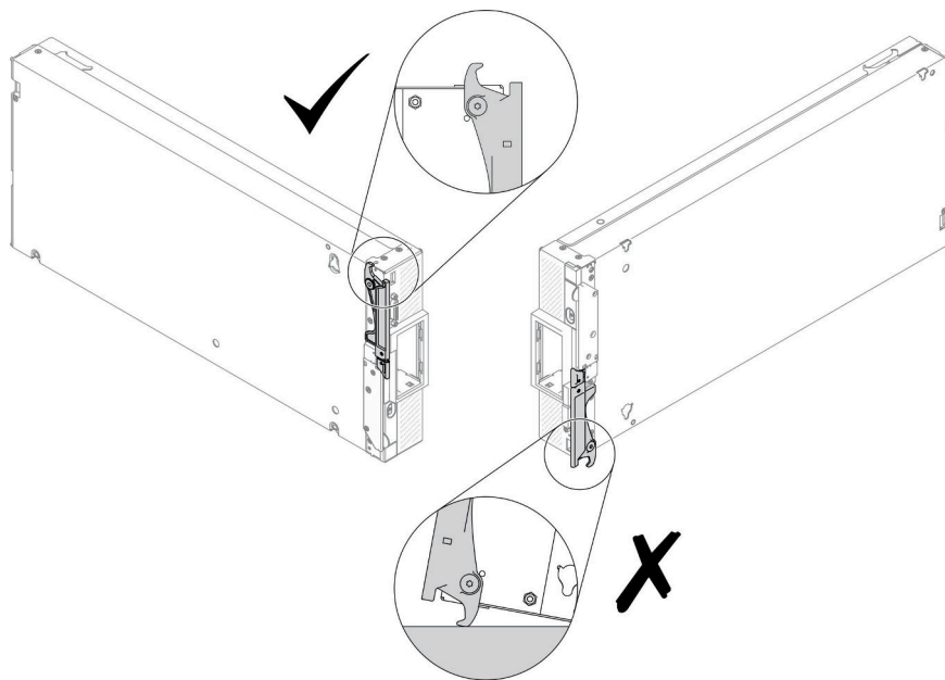
図 76. 計算ノードを置く方向
