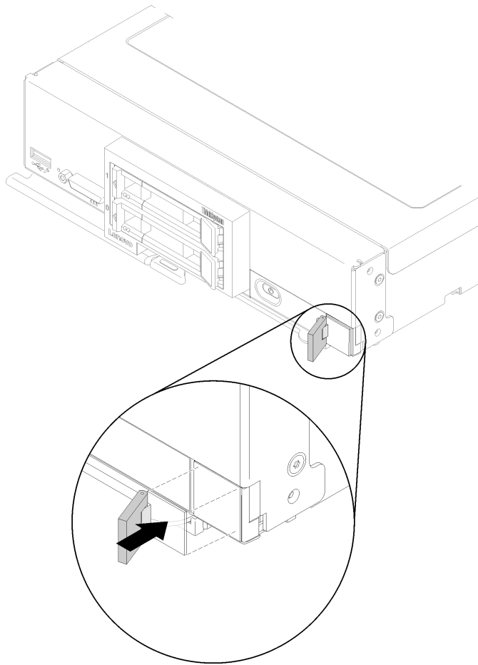
図 60. RFID タグの取り付け
