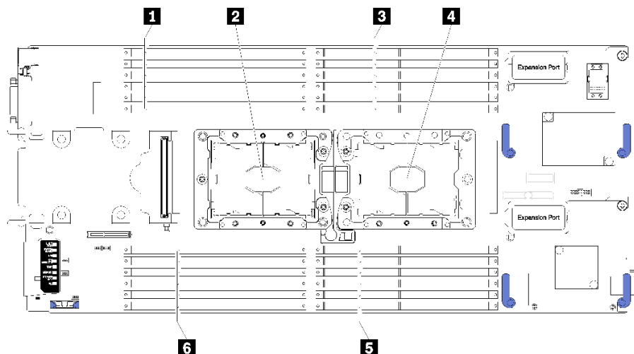
図 47. メモリー・モジュールとプロセッサの位置
