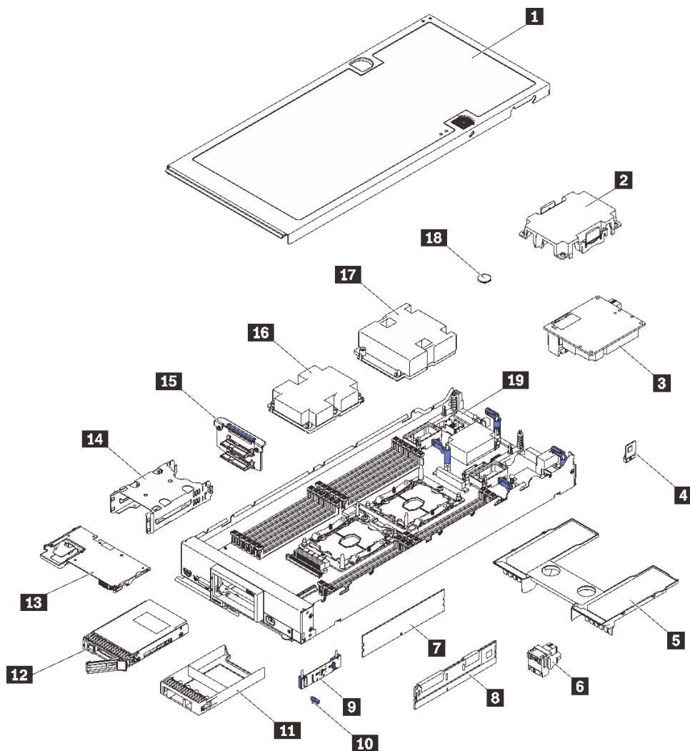
図7. 計算ノードのコンポーネント
