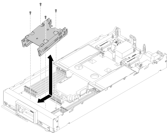
図66. ストレージ・ケージの取り付け
