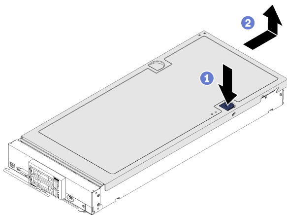
図 24. 計算ノード・カバーの取り外し
