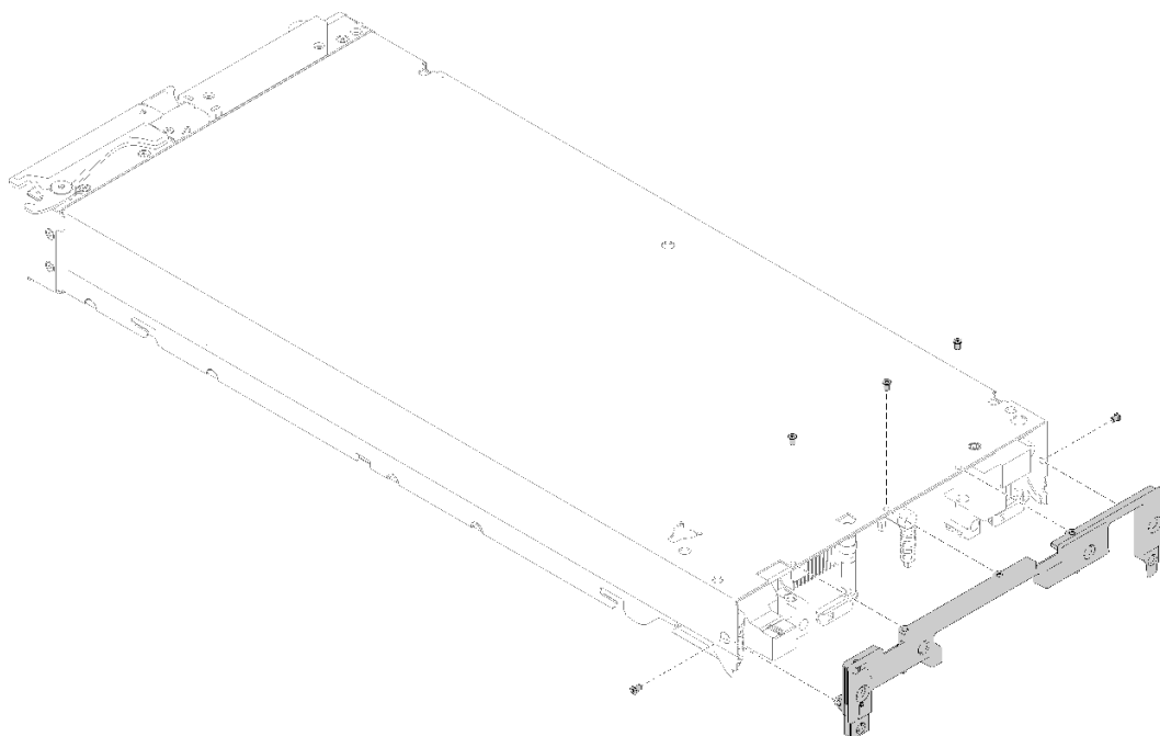
図21. バルクヘッドの取り付け
