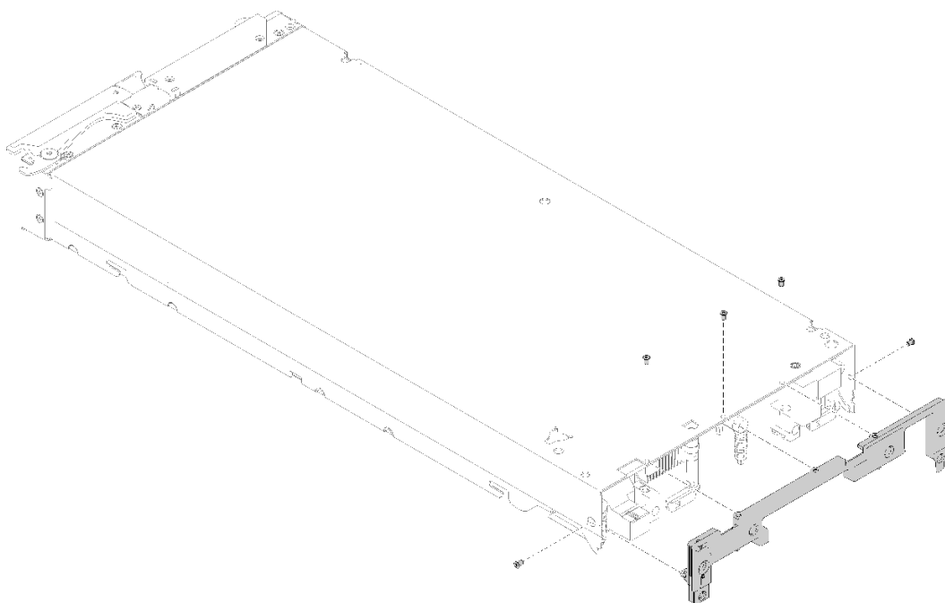
図 20. バルクヘッドの取り外し
