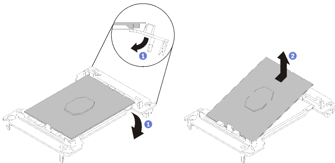
図53. プロセッサ保持器具の取り外し
