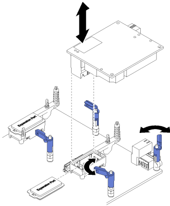
図 34. I/O 拡張アダプターの取り外し
