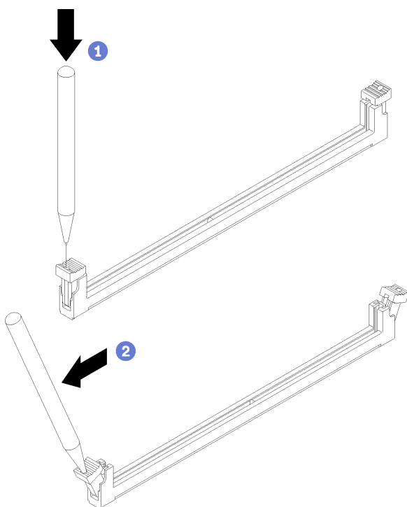
図45. 保持クリップを開く
