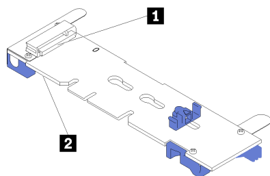
図42. M.2 ドライブ・スロット
