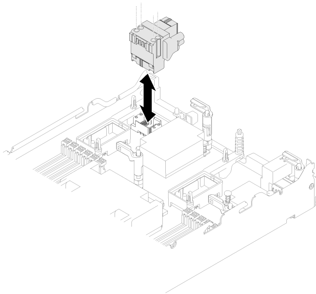
図27. ファブリック・コネクタの取り付け
