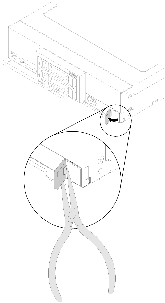
図 59. RFID タグの取り外し
