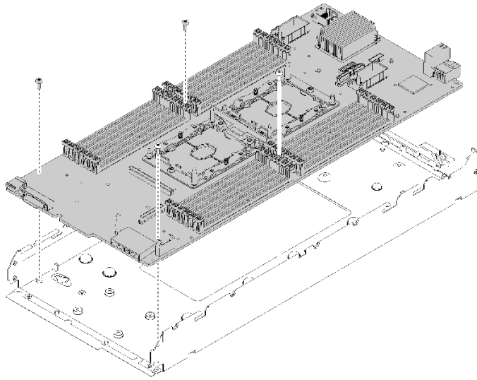
図 80. システム・ボードの取り外し
