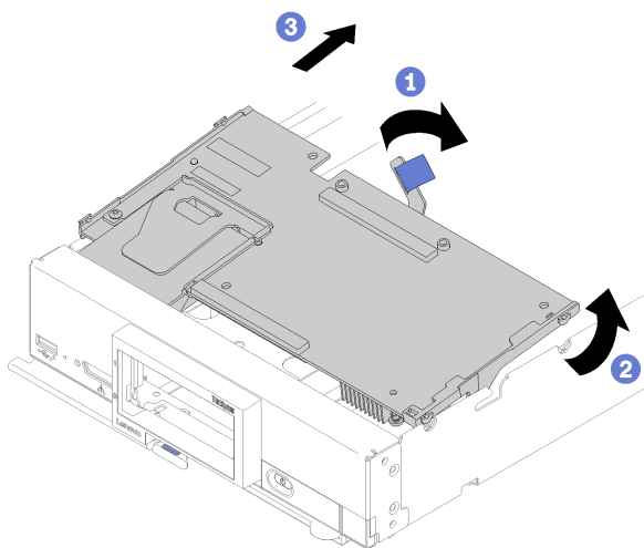
図 61. RAID アダプターの取り外し
