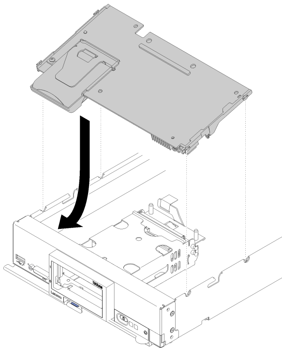
図 63. RAID アダプターの取り付け
