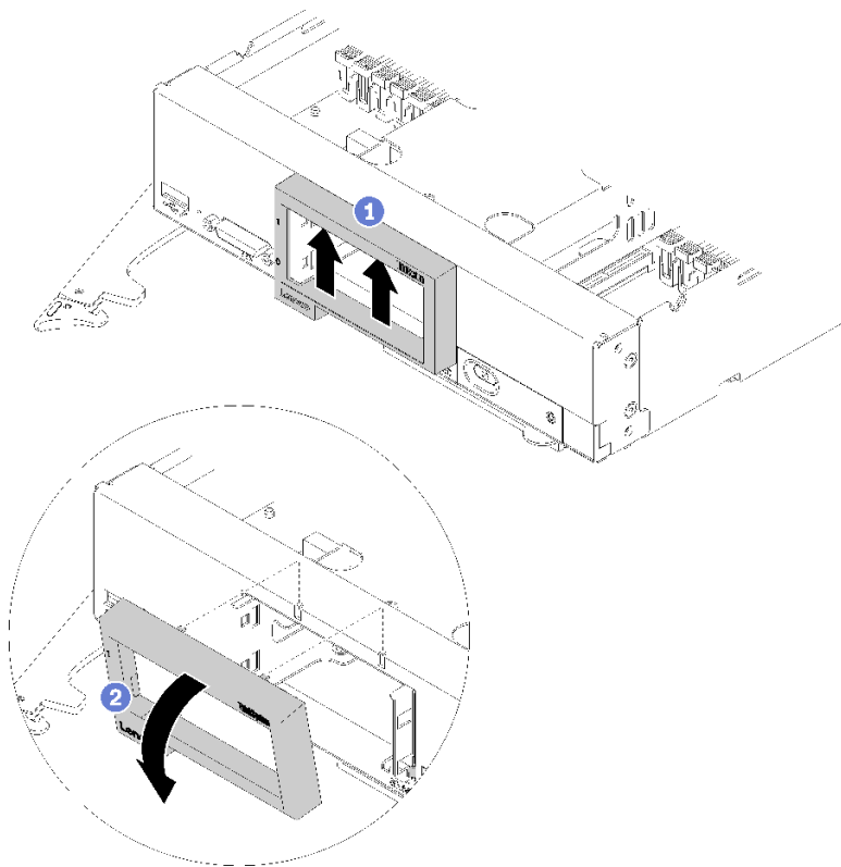
図 18. ベゼルの取り外し
