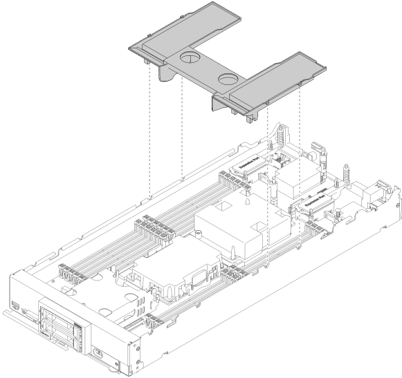
図 15. エアー・バッフルの取り付け
