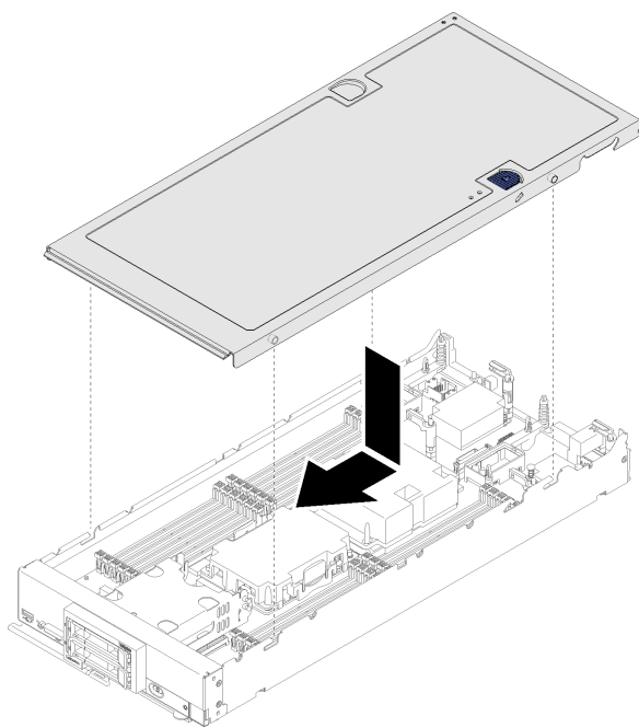
図 25. 計算ノード・カバーの取り付け
