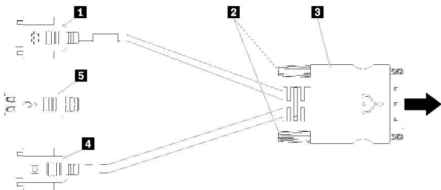
図 6. KVM ケーブルのコネクタおよびコンポーネント
