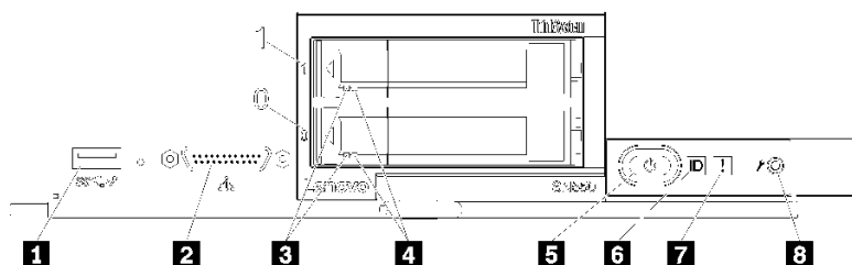
図 3. 計算ノードのコントロール・パネルのボタン、コネクタ、および LED
