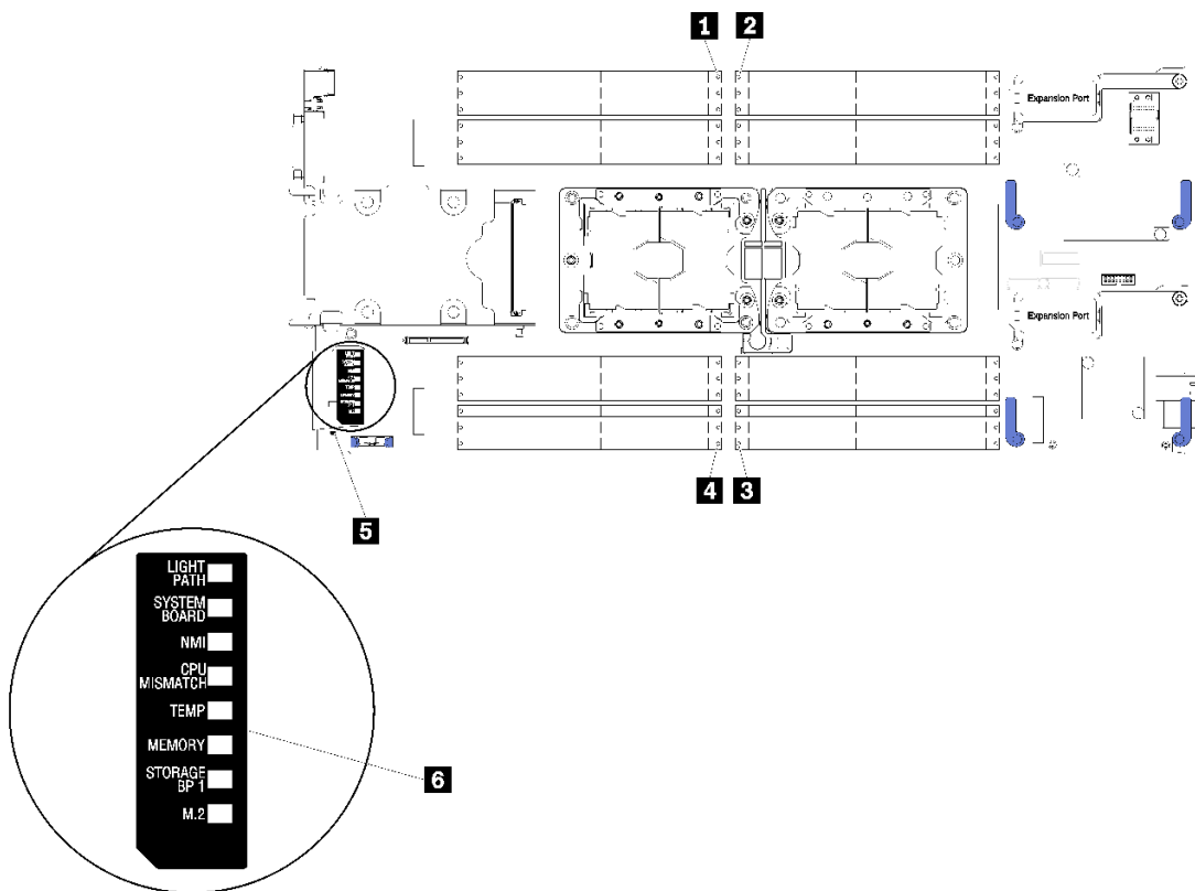
図 75. システム・ボード LED
