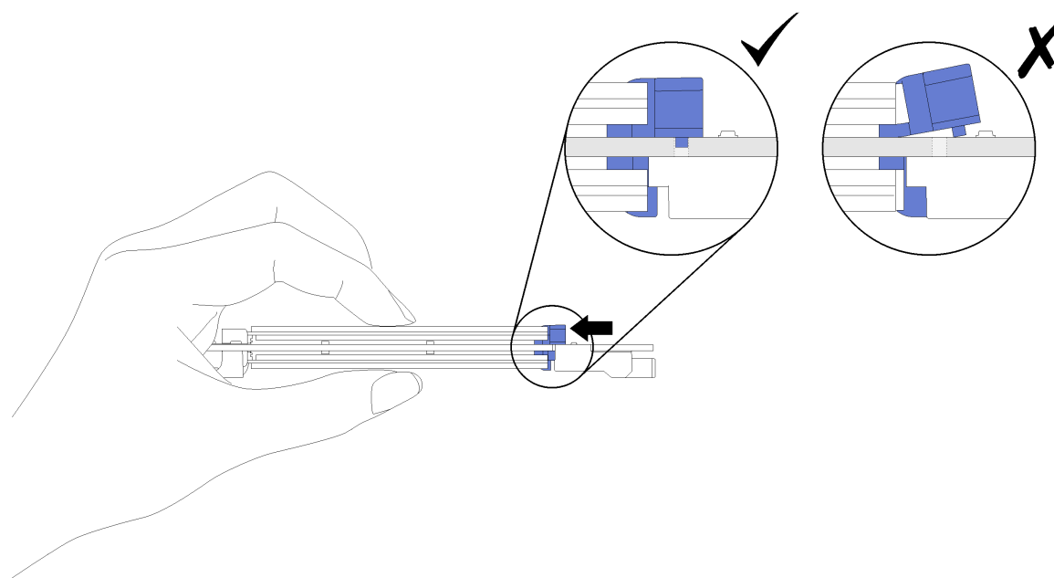
図 44. M.2 ドライブの取り付け
