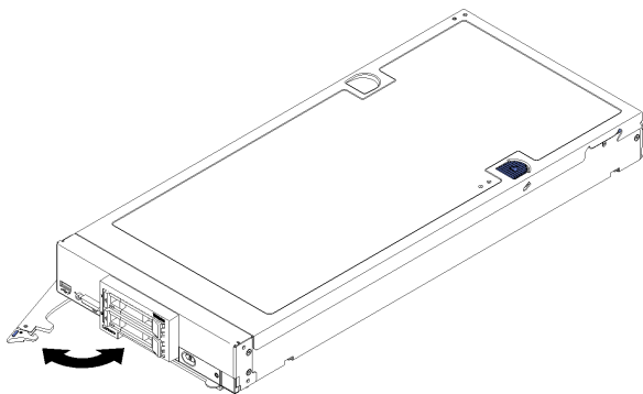
図8. シャーシからの計算ノードの取り外し
