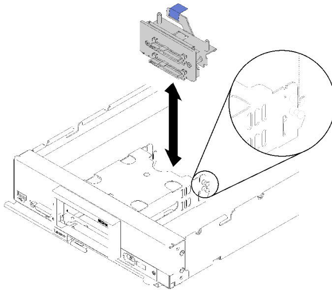
図 62. ドライブ・バックプレーンの取り付け
