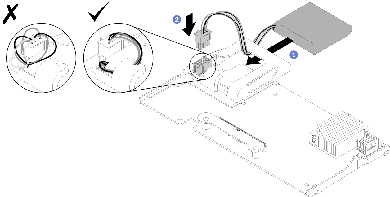
図29. フラッシュ電源モジュールの取り付け
