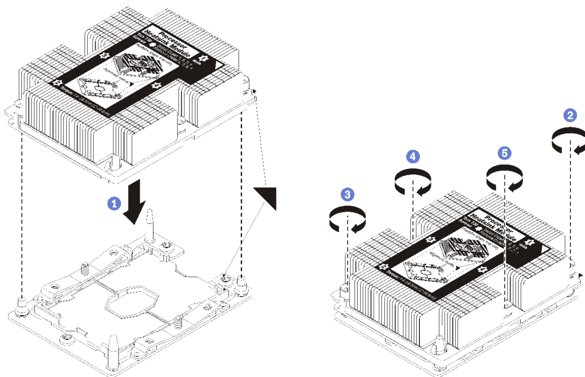
図 58. PHM の取り付け
