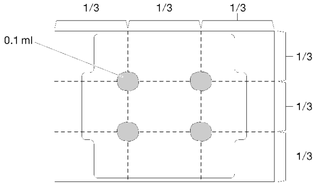
図 55. 熱伝導グリースの適切な形
