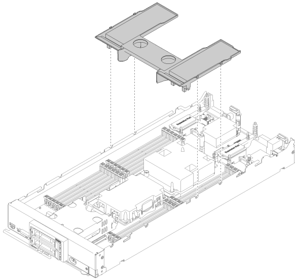
図 14. エアー・バッフルの取り外し
