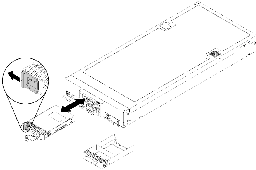
図 11. 2.5 型ホット・スワップ・ドライブの取り付け
