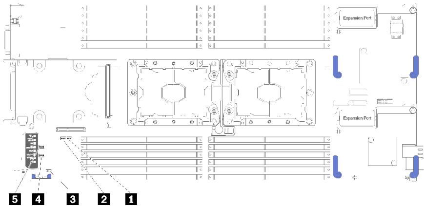
図5. システム・ボード・スイッチ
