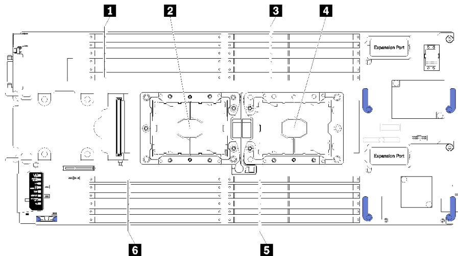
図 50. DIMM とプロセッサの位置
