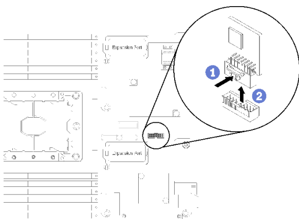
図 68. TCM/TPM アダプターの取り外し
