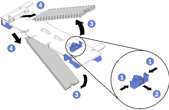
図 40. M.2 ドライブの取り外し
