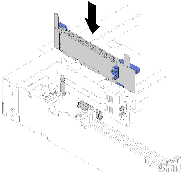
図 39. M.2 バックプレーンの取り付け
