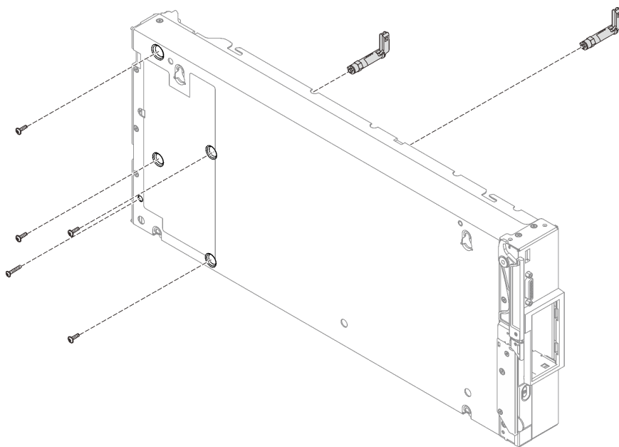
図 77. シャーシ底部からのねじの取り外し
