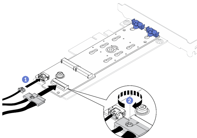
図 49. 電源および信号ケーブルの接続
