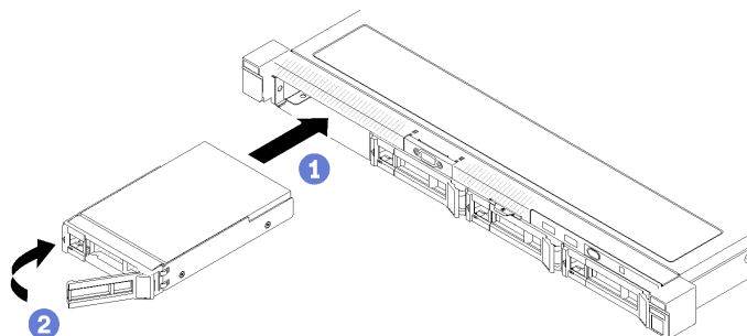
図 69. 3.5 型ホット・スワップ・ドライブの取り付け
