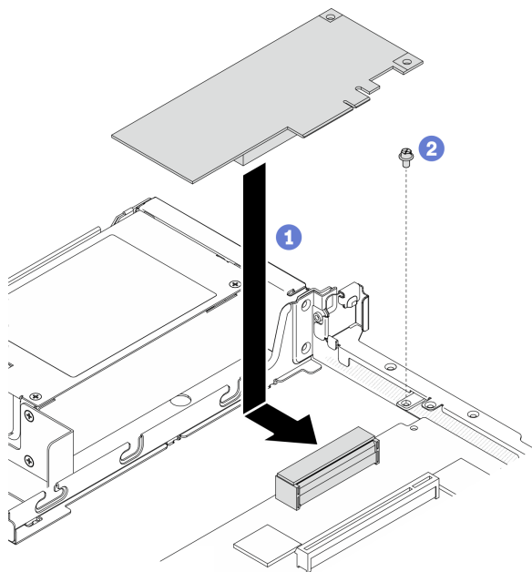
図 53. PCIe アダプターの取り付け
