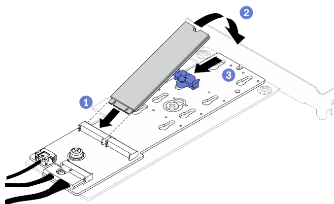
図 51. M.2 ドライブの取り付け
