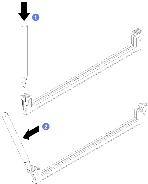
図 57. 保持クリップを開く
