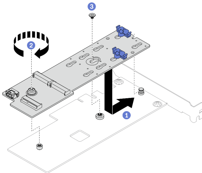
図 48. M.2 ブート・アダプターの取り付け
