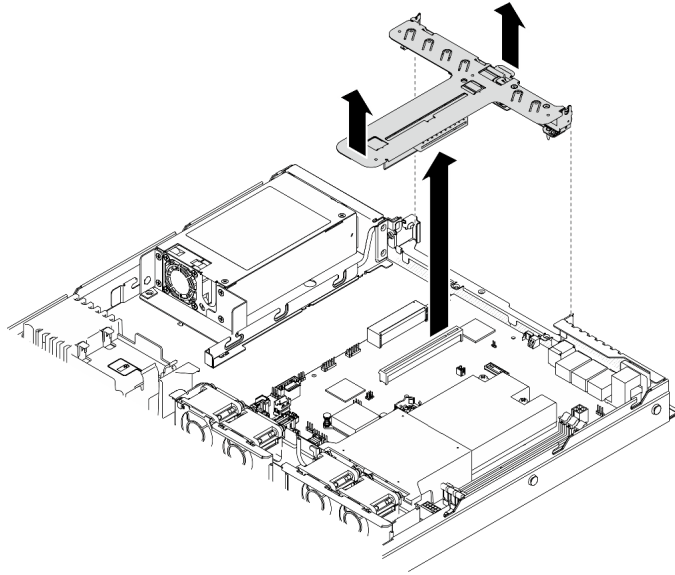
図 47. PCIe ライザー・アセンブリーの取り外し
