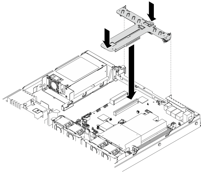
図 54. PCIe ライザー・アセンブリーの取り付け
