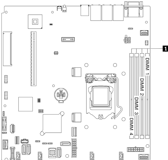
図 44. システム・ボードのメモリー・モジュール・スロットの位置
