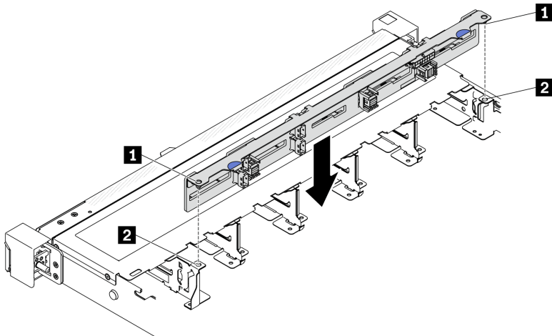
図 59. 2.5 型バックプレーンの取り付け
