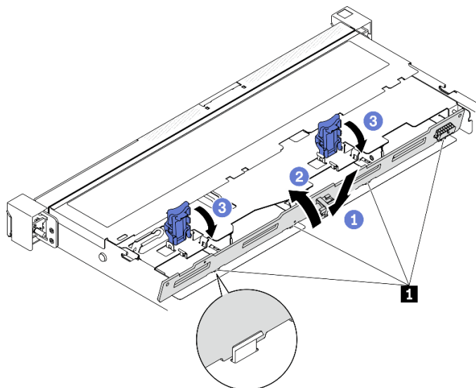
図 60. 3.5 型バックプレートの取り付け
