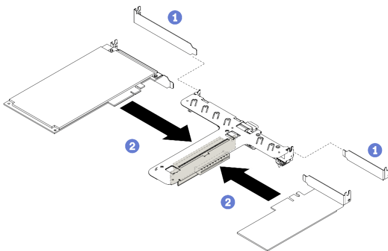
図 52. PCIe アダプターの取り付け
