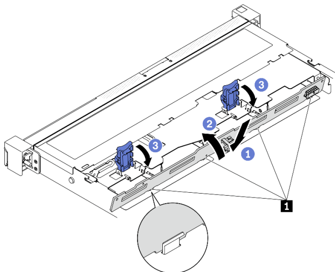
図 61. バックプレートの取り付け
