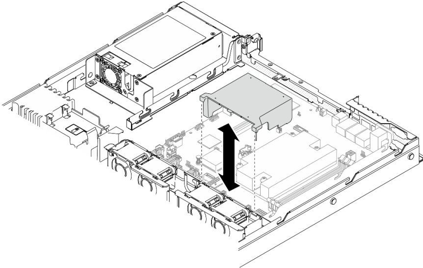
図 46. エア・バッフルの取り外し
