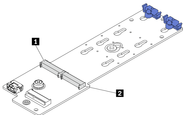
図 50. M.2 ドライブ・スロット
