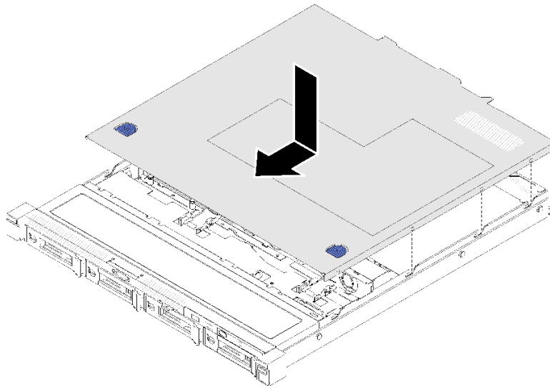
図 63. トップ・カバーの取り付け
