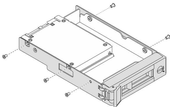
図 66. 2.5 型ドライブおよびドライブ・アダプターを固定するねじの取り付け
