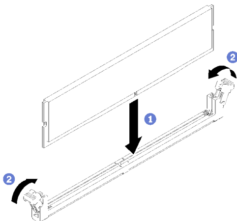
図58. メモリー・モジュールの取り付け
