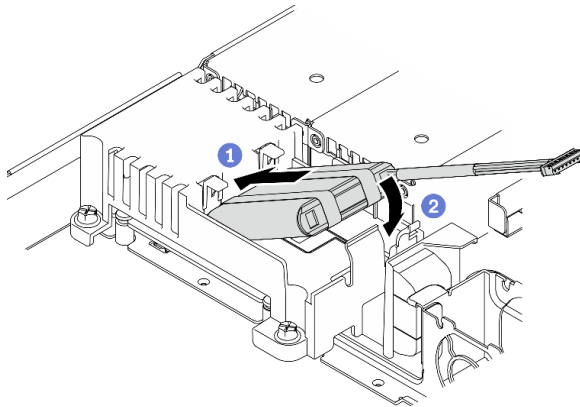
図 55. フラッシュ電源モジュールの取り付け
