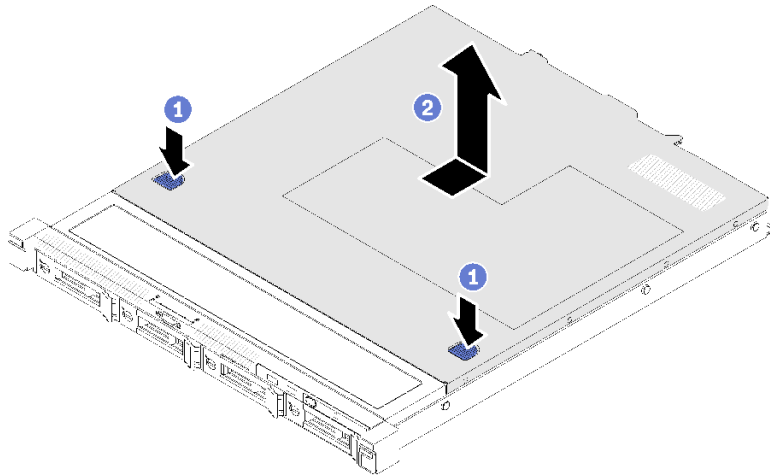
図 45. トップ・カバーの取り外し
