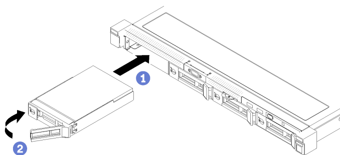
図 67. シンプル・スワップ・ドライブの取り付け
