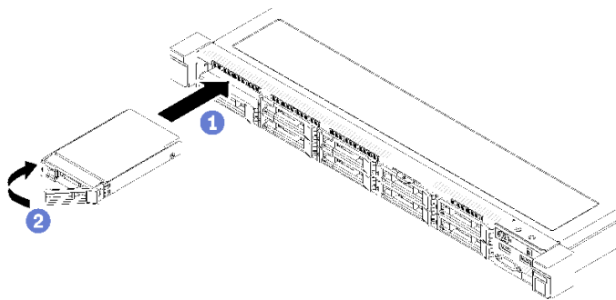
図 68. 2.5 型ホット・スワップ・ドライブの取り付け
