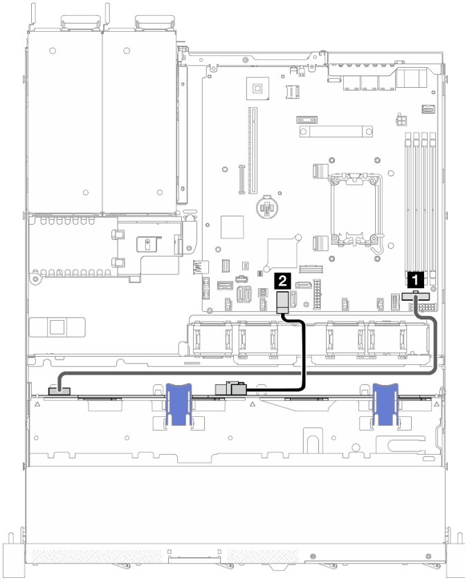
Figure 142. Quatre unités SATA/SAS (logiciel RAID)
