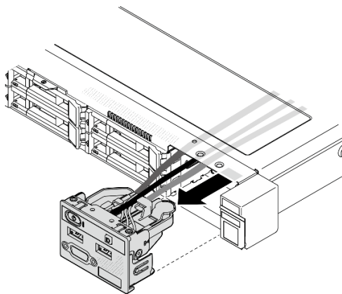
Figure 35. Retrait du module d'E-S avant
