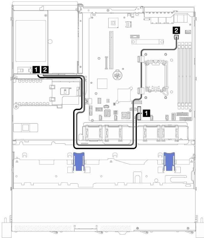
Figure 132. Cheminement des câbles de l'unité d'alimentation fixe
