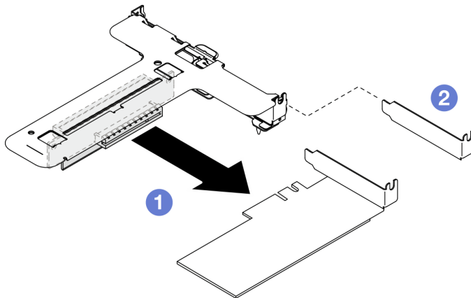
Figure 67. Retrait d'un adaptateur PCIe (emplacement 1)
