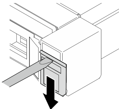
Figure 98. Retrait de l'étiquette d'identification
