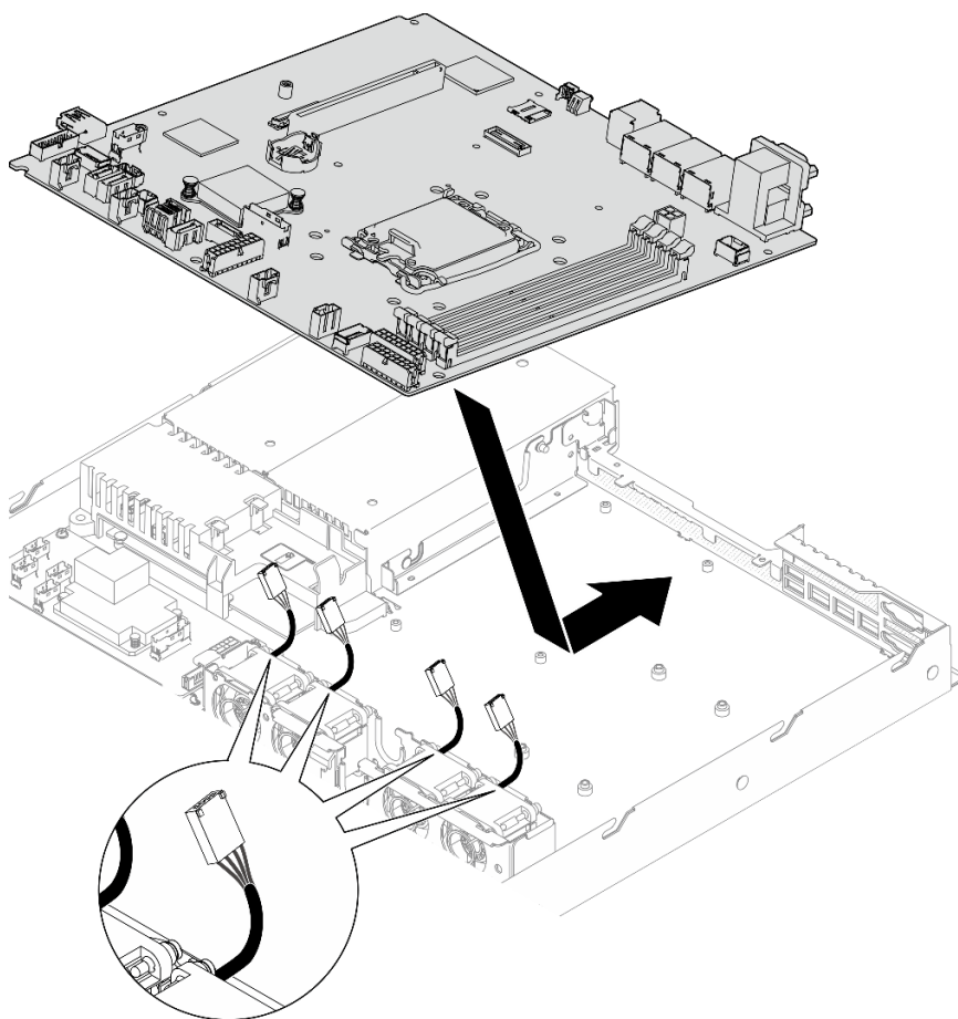
Figure 112. Installation de la carte mère
