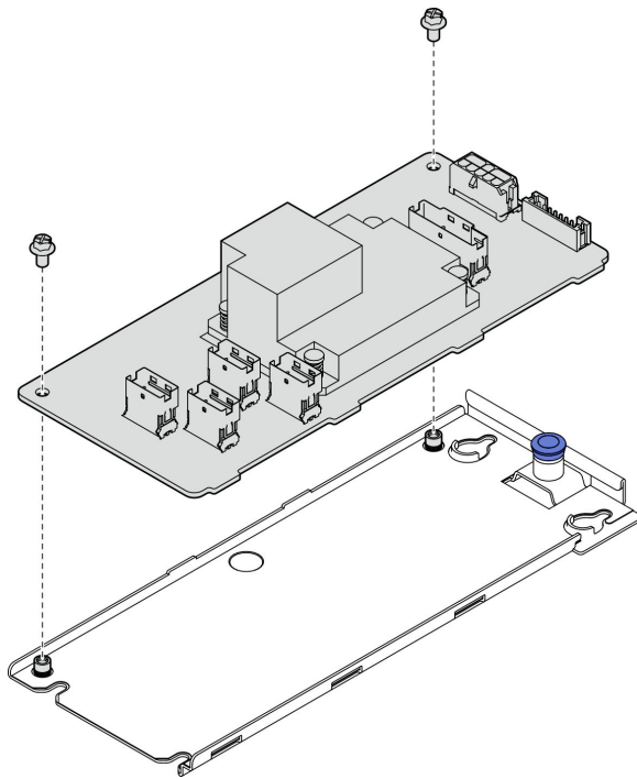
Figure 18. Installation du plateau de l'adaptateur CFF interne
