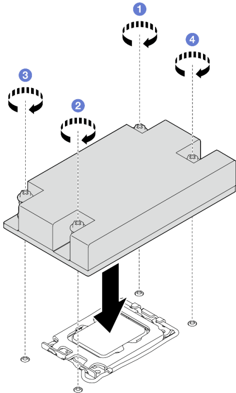
Figure 43. Installation du dissipateur thermique
