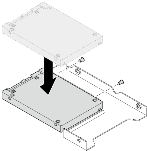
Figure 8. Installation d'une unité 2,5 pouces dans un adaptateur d'unité
