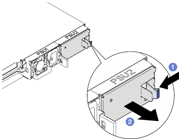
Figure 84. Retrait de l'obturateur de PSU
