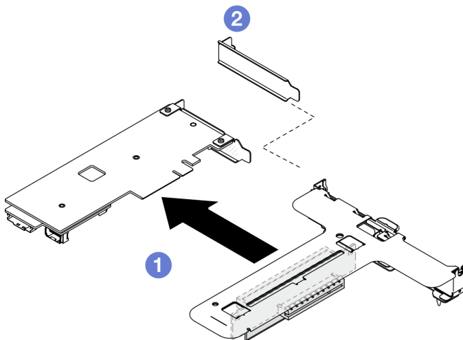
Figure 68. Retrait d'un adaptateur PCIe (emplacement 2)
