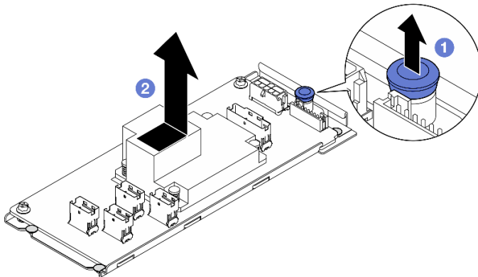
Figure 16. Retrait de l'adaptateur CFF interne
