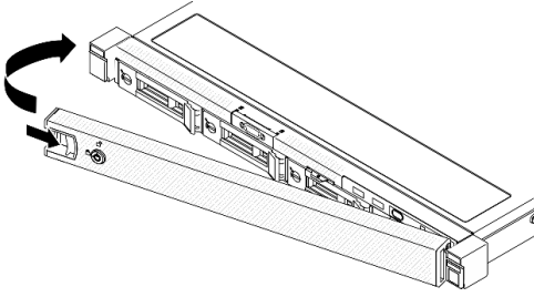
Figure 106. Installation du panneau de sécurité
