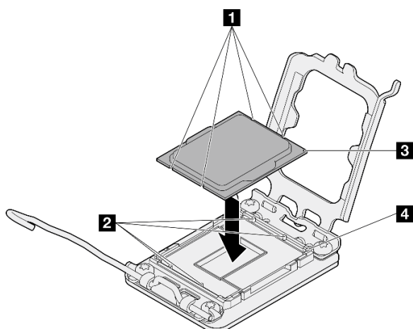
Figure 95. Installation du processeur
