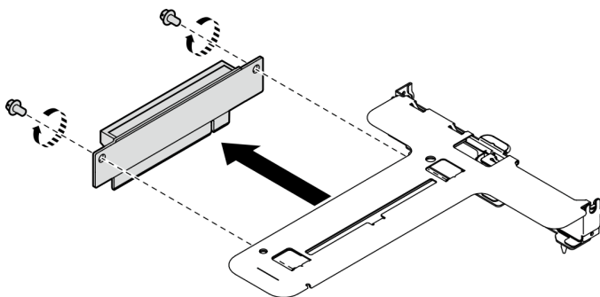
Figure 66. Retrait d'une carte mezzanine PCIe
