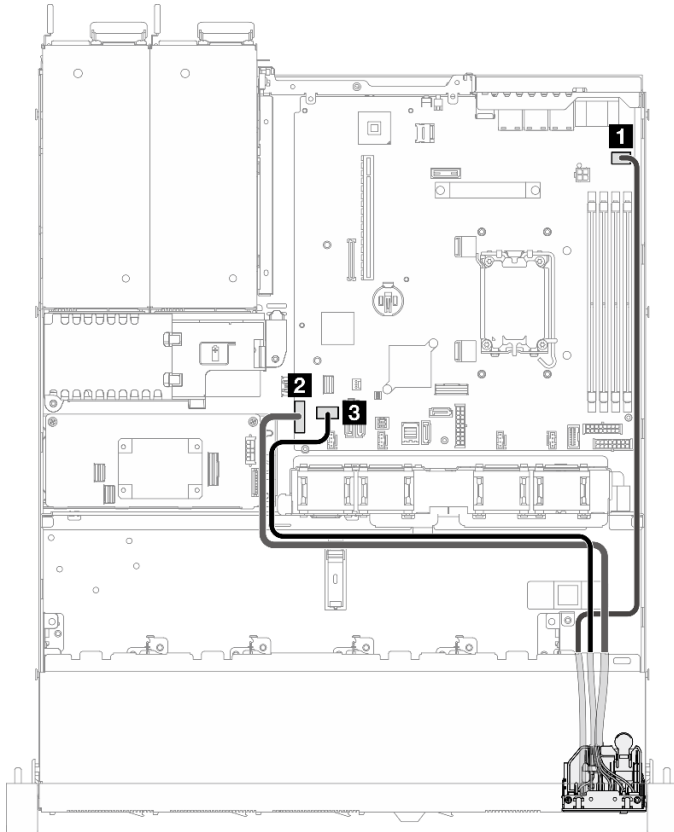
Figure 130. Cheminement des câbles du module d'E-S avant pour modèle 2,5 pouces
