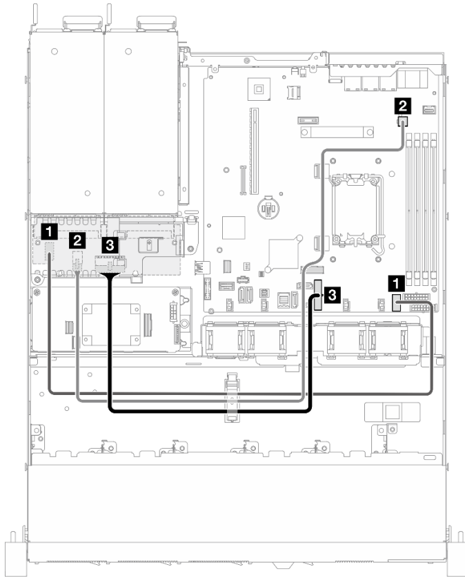
Figure 133. Cheminement des câbles du tableau de distribution
