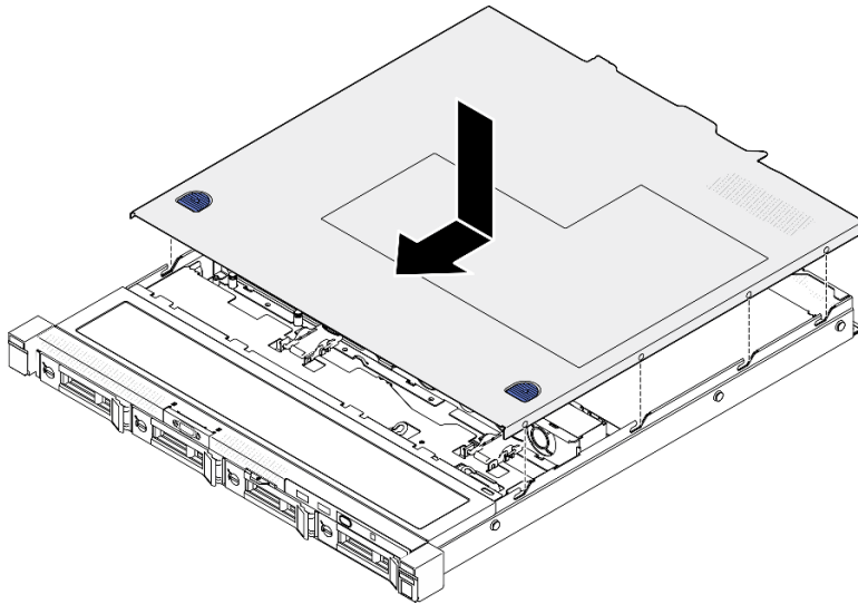
Figure 115. Installation du carter supérieur
