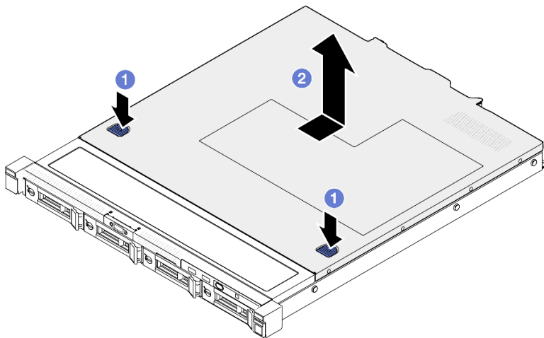
Figure 114. Retrait du carter supérieur
