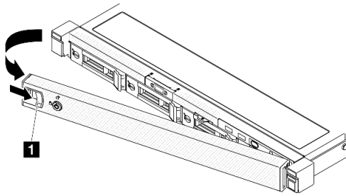
Figure 105. Retrait du panneau de sécurité
