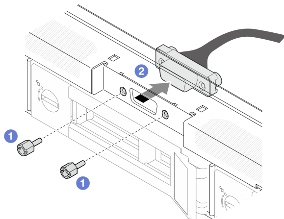
Figure 119. Retrait du câble VGA
