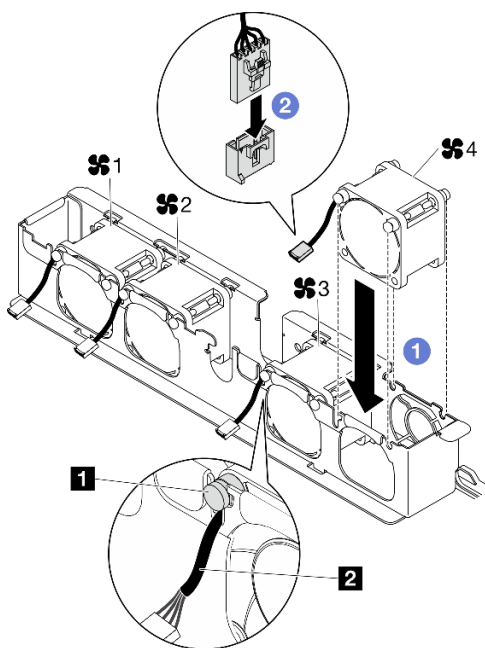
Figure 31. Installation du ventilateur
