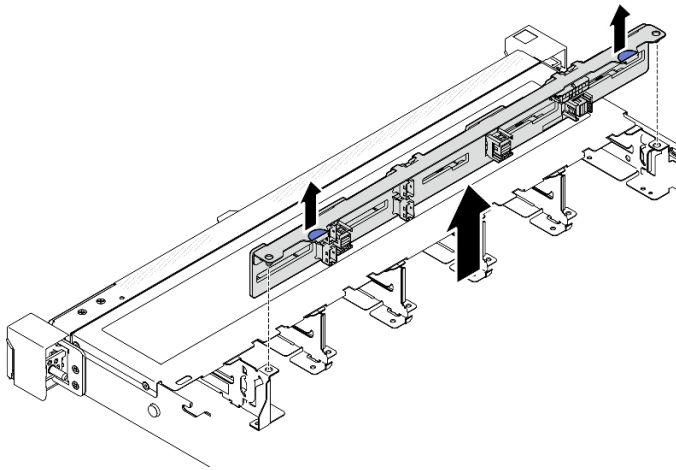
Figure 2. Retrait de dix fonds de panier d'unité remplaçable à chaud 2,5 pouces
