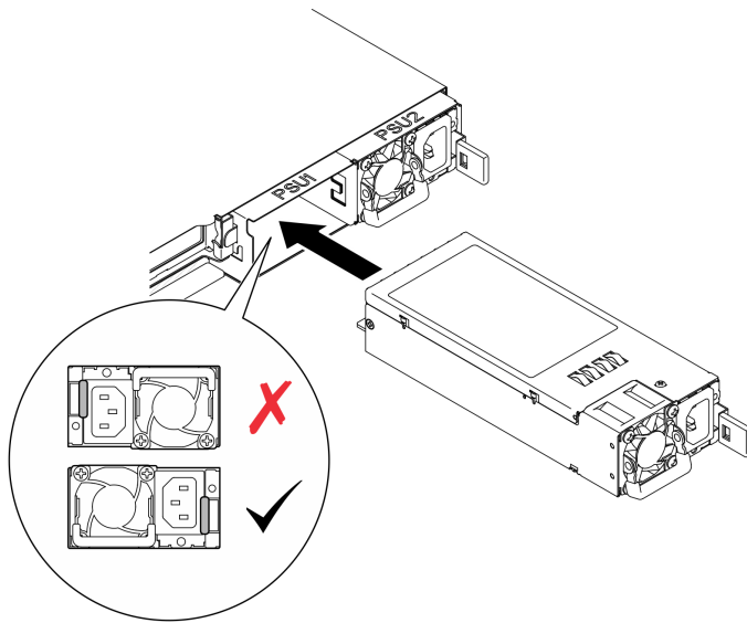
Figure 85. Installation de l'unité d'alimentation remplaçable à chaud
