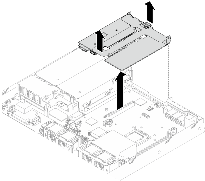
Figure 65. Retrait de l'assemblage de cartes mezzanines PCIe
