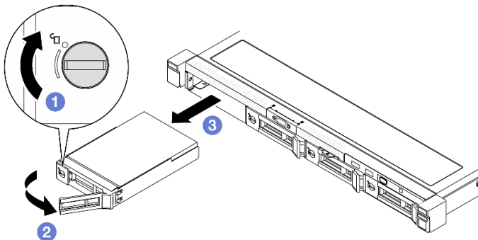
Figure 24. Retrait d'une unité à remplacement standard
