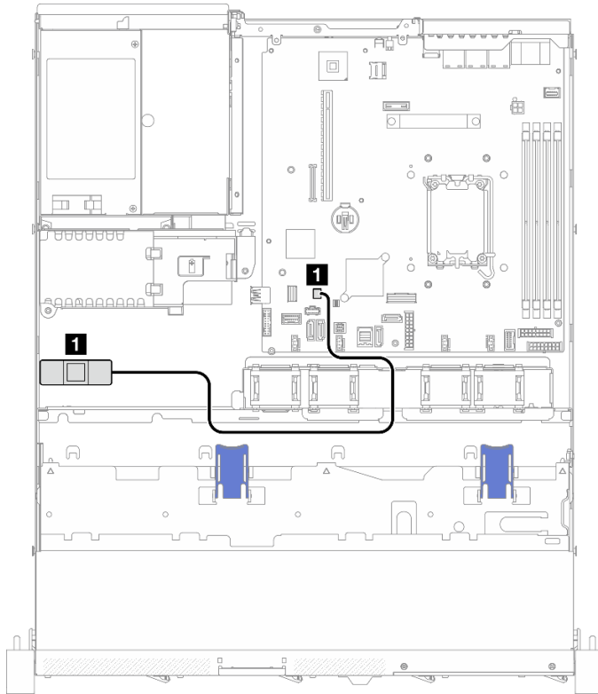
Figure 135. Acheminement des câbles du commutateur d'intrusion pour un modèle 3,5 pouces
