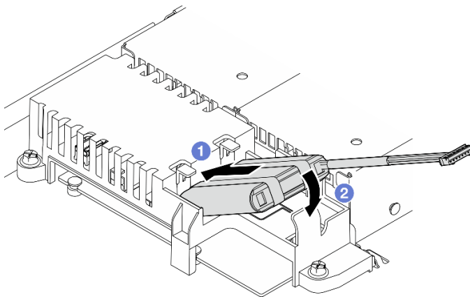
Figure 33. Installation du module d'alimentation flash
