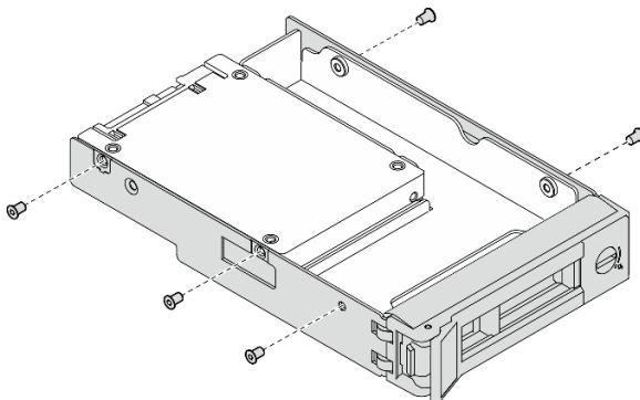
Figure 9. Installation des vis sur l'adaptateur d'unité
