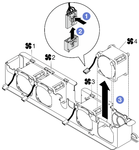
Figure 30. Retrait du ventilateur
