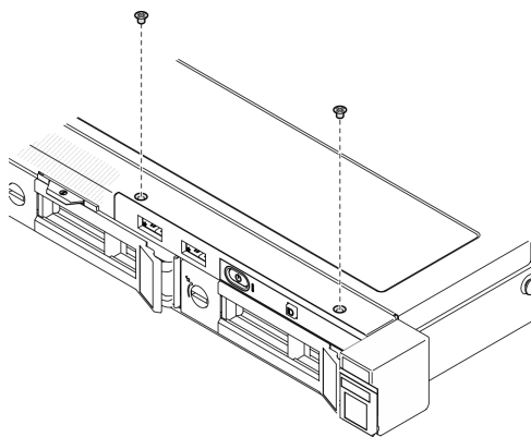
Figure 41. Installation du module d'E-S avant
