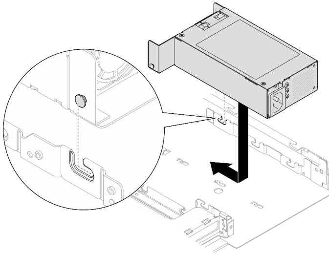
Figure 78. Installation du bloc d'alimentation fixe
