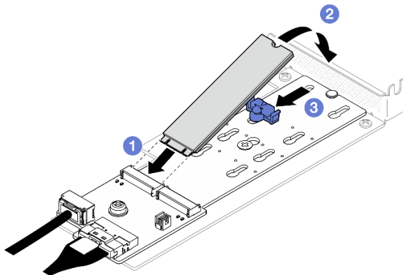
Figure 60. Installation d'une unité M.2
