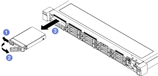
Figure 26. Retrait d'une unité remplaçable à chaud 2,5 pouces
