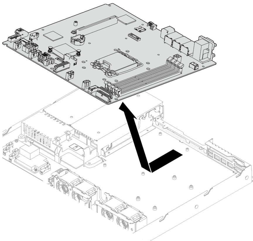
Figure 111. Retrait de la carte mère
