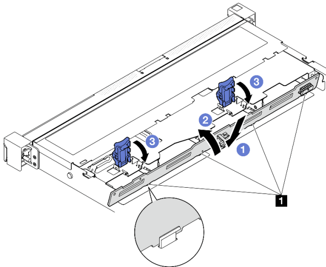
Figure 11. Installation du fond de panier 3,5 pouces
