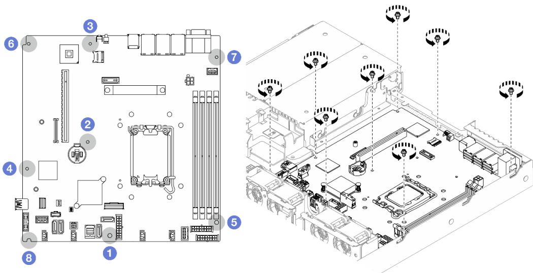
Figure 110. Emplacement des vis sur la carte mère
