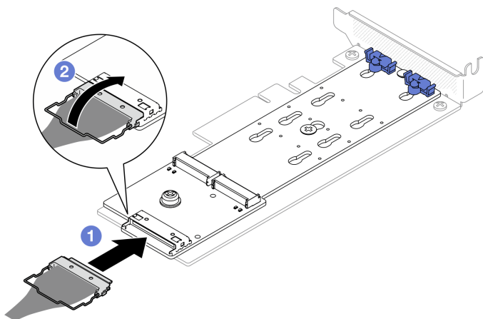
Figure 58. Connexion du câble à l'adaptateur d'amorçage SATA/NVMe M.2
