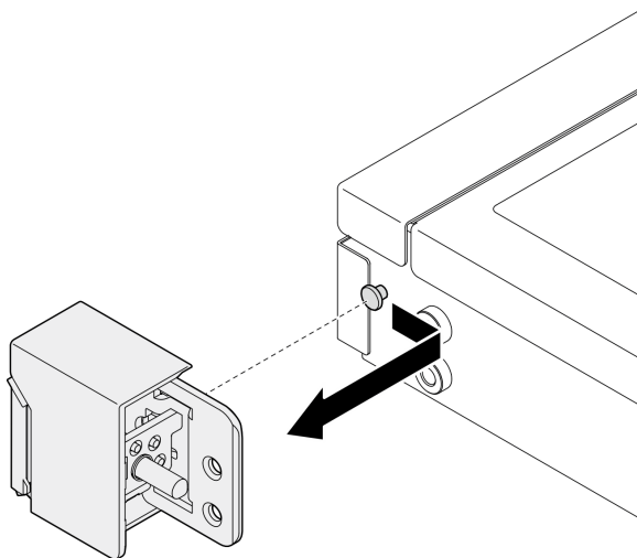
Figure 100. Retrait des taquets d'armoire
