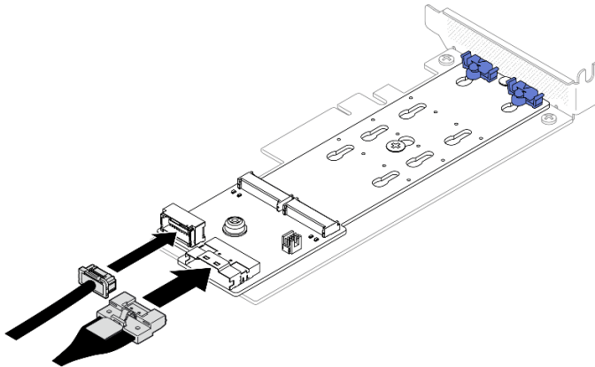
Figure 57. Connexion du câble à l'adaptateur d'amorçage SATA/x4 NVMe M.2
