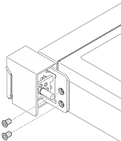
Figure 102. Installation des taquets d'armoire
