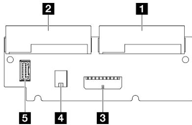
Figure 127. Connecteurs du tableau de distribution
