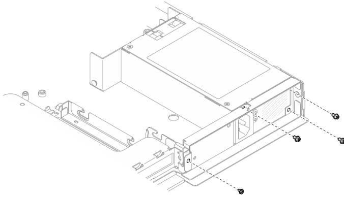
Figure 75. Retrait des vis du support arrière
