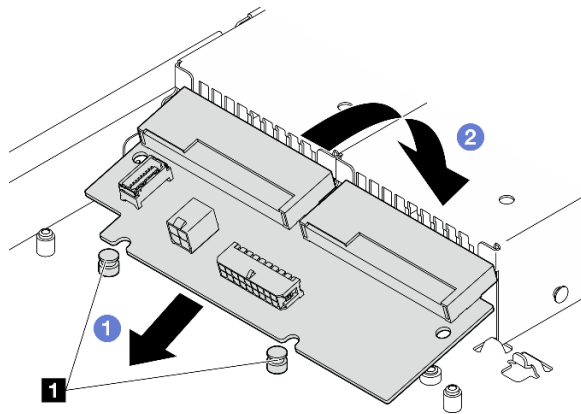
Figure 90. Installation du tableau de distribution
