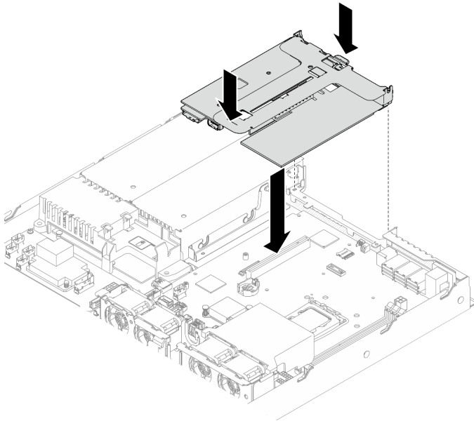
Figure 72. Installation de l'assemblage de cartes mezzanines PCIe
