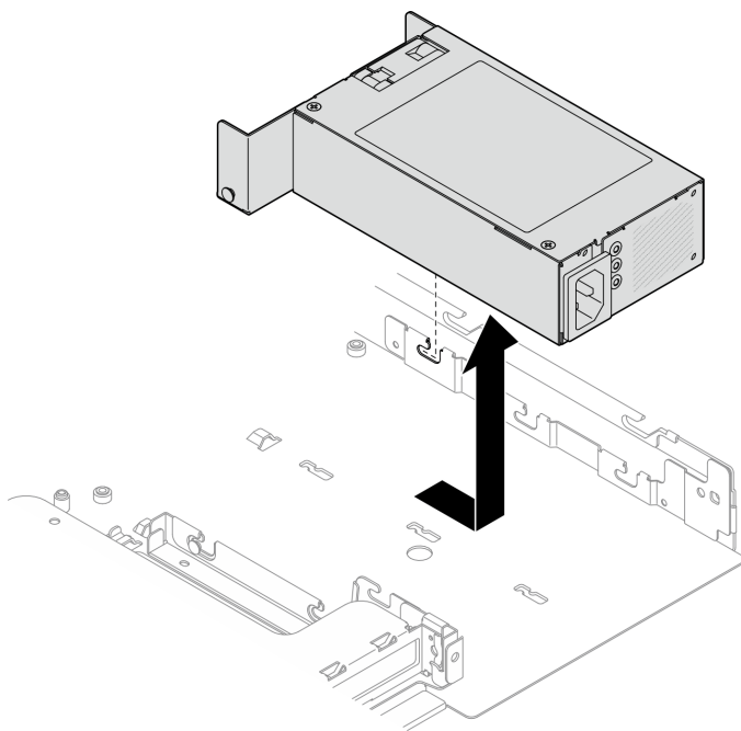
Figure 77. Retrait du bloc d'alimentation fixe
