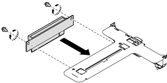
Figure 71. Installation d'une carte mezzanine PCIe
