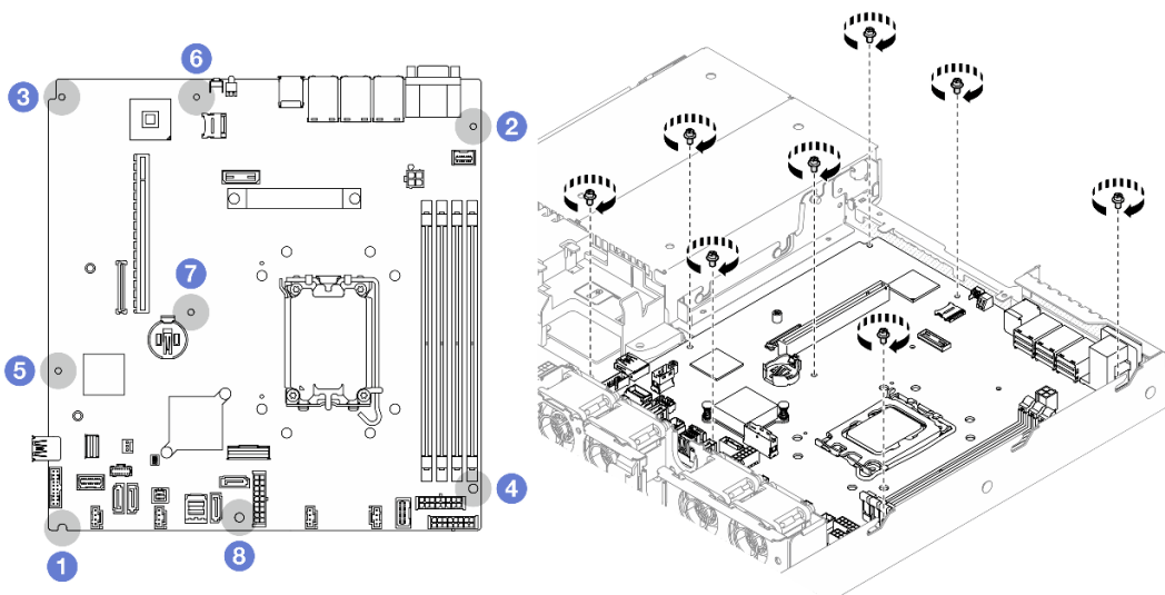
Figure 113. Emplacement des vis sur la carte mère
