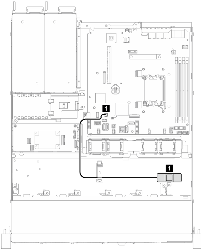
Figure 136. Acheminement des câbles du commutateur d'intrusion pour un modèle 2,5 pouces
