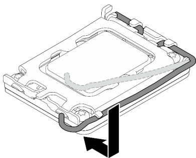
Figure 96. Fermeture du dispositif de retenue du processeur
