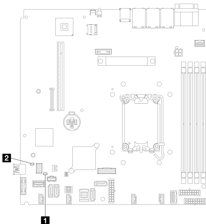
Figure 158. Voyants de la carte mère
