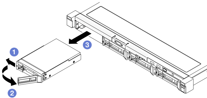
Figure 27. Retrait d'une unité remplaçable à chaud 3,5 pouces
