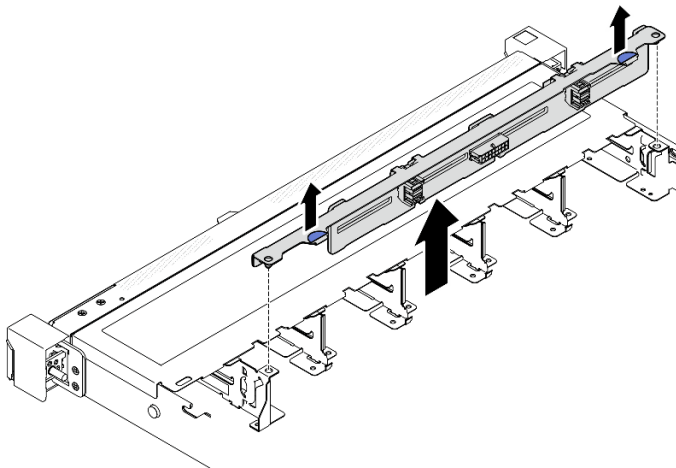
Figure 3. Retrait de huit fonds de panier d'unité remplaçable à chaud 2,5 pouces
