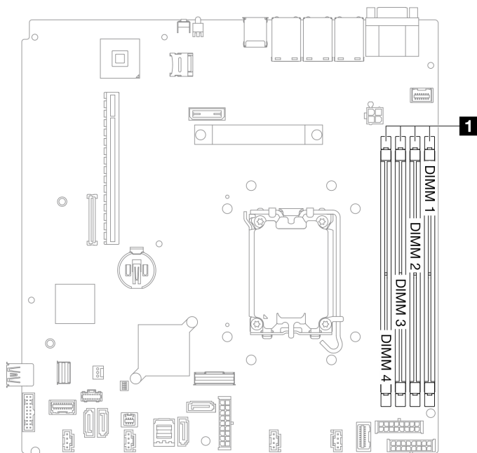
1 Emplacements de module de mémoire
