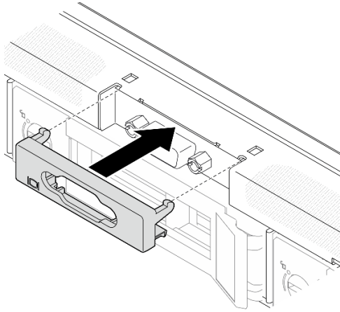
Figure 121. Installation du cache de la barrette VGA
