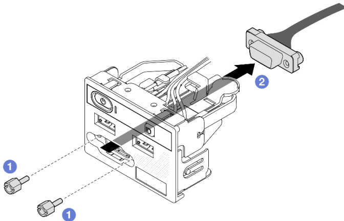
Figure 116. Retrait du câble VGA
