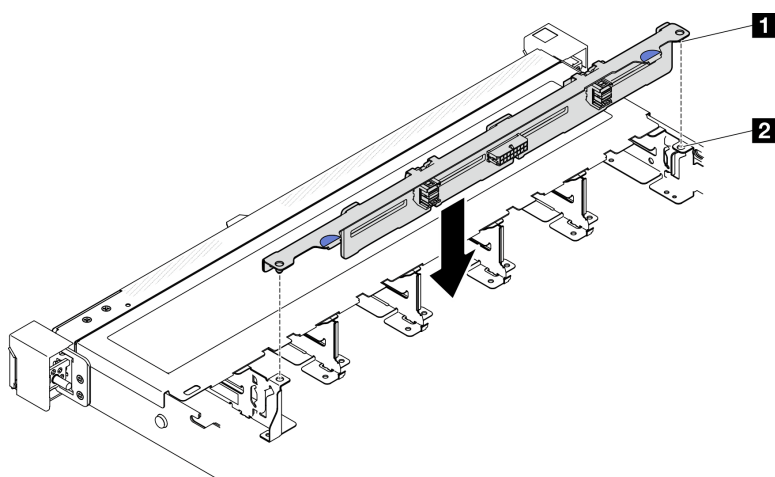
Figure 5. Installation de huit fonds de panier d'unité remplaçable à chaud 2,5 pouces
