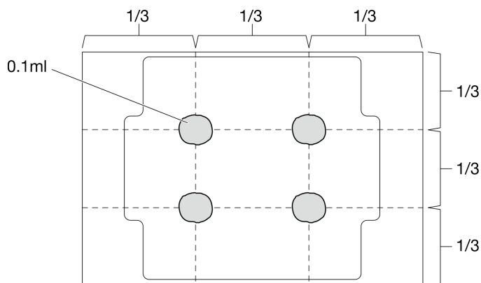
Figure 97. Forme correcte de la pâte thermoconductrice
