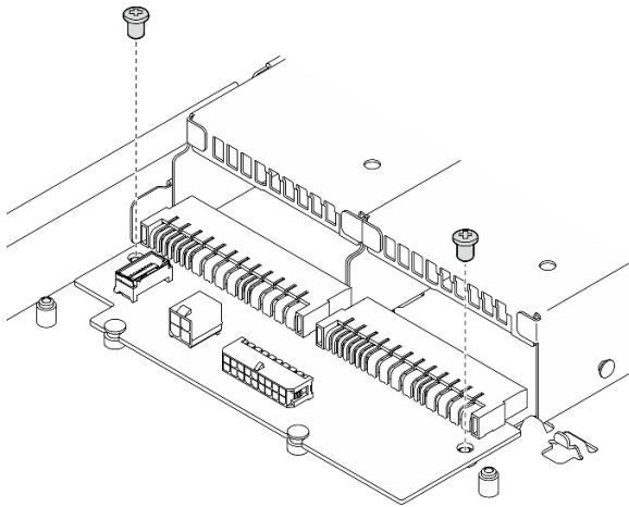
Figure 88. Retrait de la vis du tableau de distribution d'alimentation
