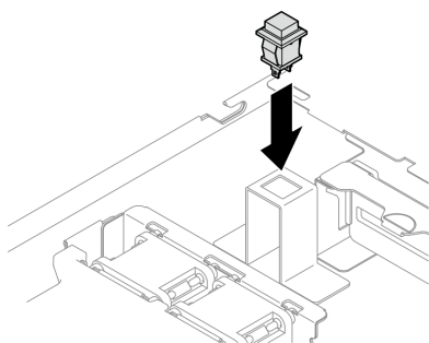
Figure 49. Installer le commutateur de détection d'intrusion
