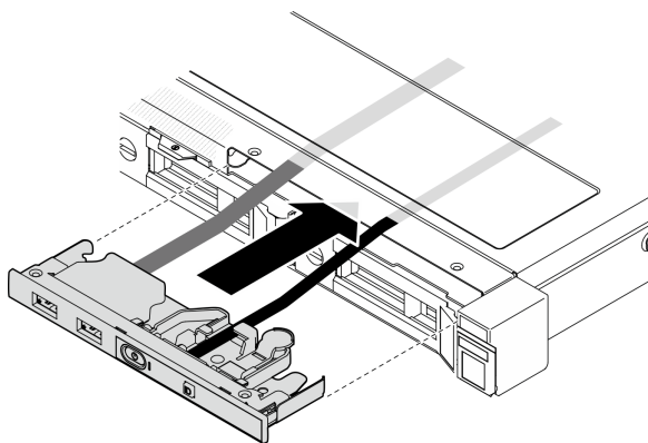
Figure 40. Installation du module d'E-S avant
