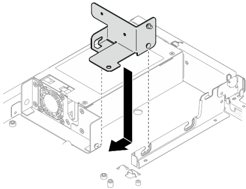
Figure 81. Installation du support du bloc d'alimentation
