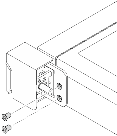
Figure 99. Retrait des taquets d'armoire
