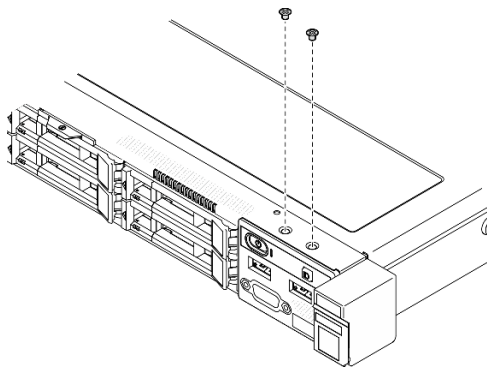
Figure 34. Retrait des vis du module d'E-S avant
