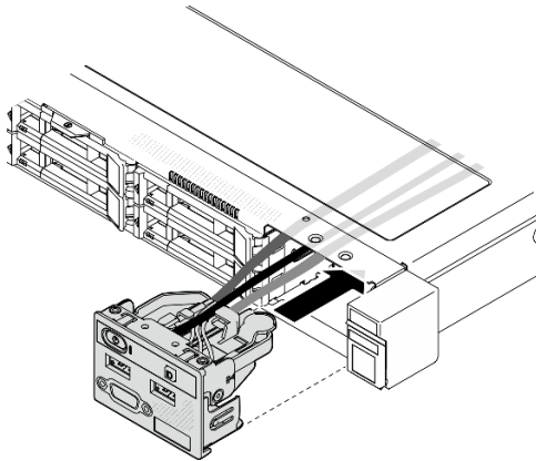
Figure 36. Installation du module d'E-S avant (modèle d'unité 2,5 pouces)
