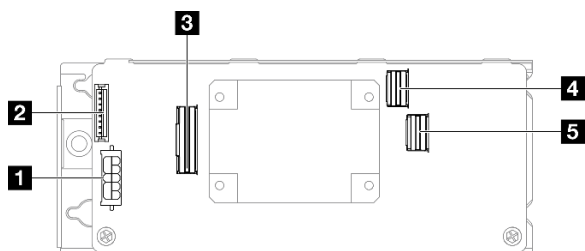
Figure 122. Connecteurs de l'adaptateur RAID 8i CFF
