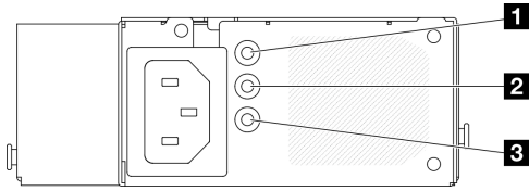
Figure 156. LED du bloc d'alimentation fixe
