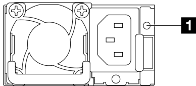
Figure 157. LED d'unité de bloc d'alimentation remplaçable à chaud
