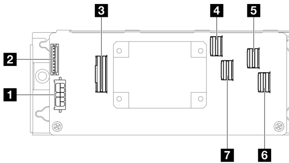
Figure 123. Connecteurs de l'adaptateur RAID 16i CFF
