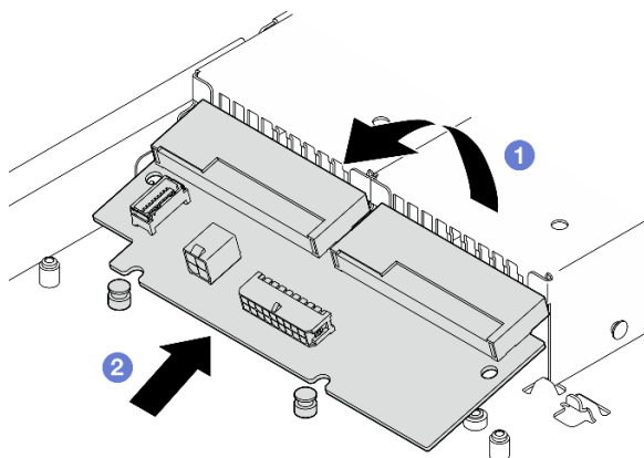
Figure 89. Tableau de distribution, retrait
