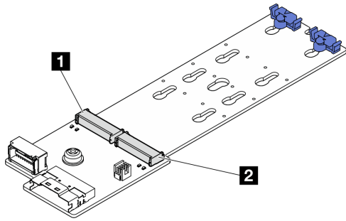
Figure 59. Emplacement de l'unité M.2
