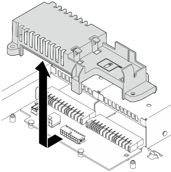
Figure 87. Retrait du carter du tableau de distribution
