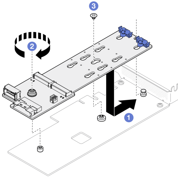
Figure 56. Installation de l'adaptateur d'amorçage M.2
