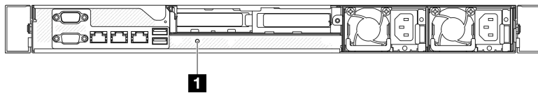
Figure 155. Voyants arrière du système
