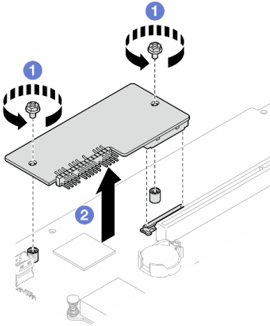
Figure 108. Retrait du module de microprogramme et de sécurité RoT
