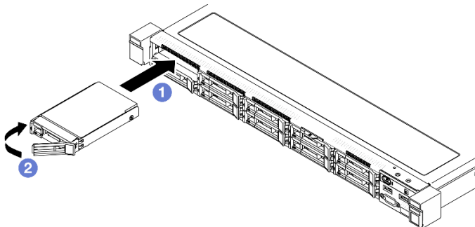
Figure 28. Installation d'une unité remplaçable à chaud 2,5 pouces
