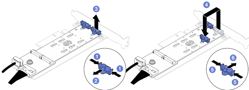
Figure 54. Ajustez le crochet de retenue M.2
