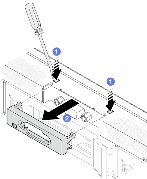
Figure 118. Retrait du cache de la barrette VGA
