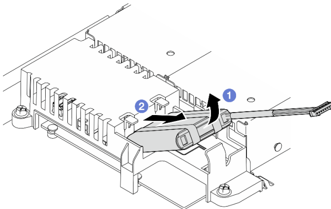
Figure 32. Retrait du module d'alimentation flash
