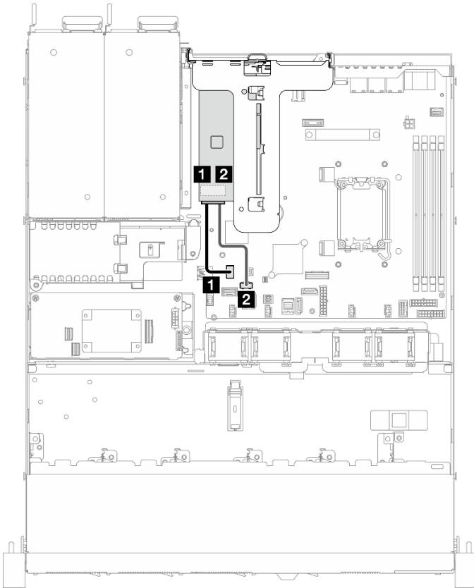
Figure 138. Cheminement des câbles pour l'adaptateur d'amorçage SATA/NVMe M.2
