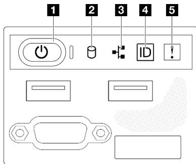
Figure 153. Module d'E-S avant sur châssis d'unité 2,5 pouces
