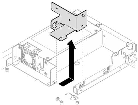
Figure 74. Retrait du support du bloc d'alimentation
