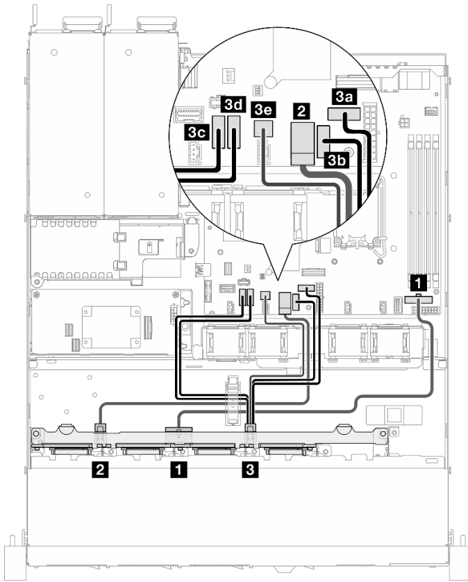
Figure 144. Huit unités SATA/SAS (logiciel RAID)
