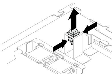
Figure 46. Retirer le commutateur de détection d'intrusion
