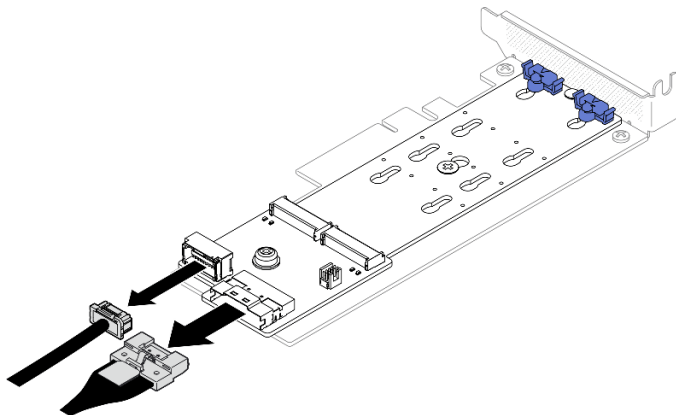
Figure 51. Déconnexion du câble de l'adaptateur d'amorçage SATA/x4 NVMe M.2
