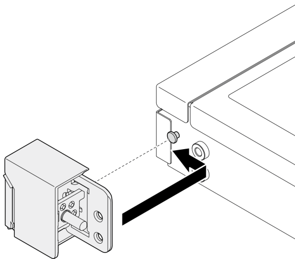
Figure 101. Installation des taquets d'armoire
