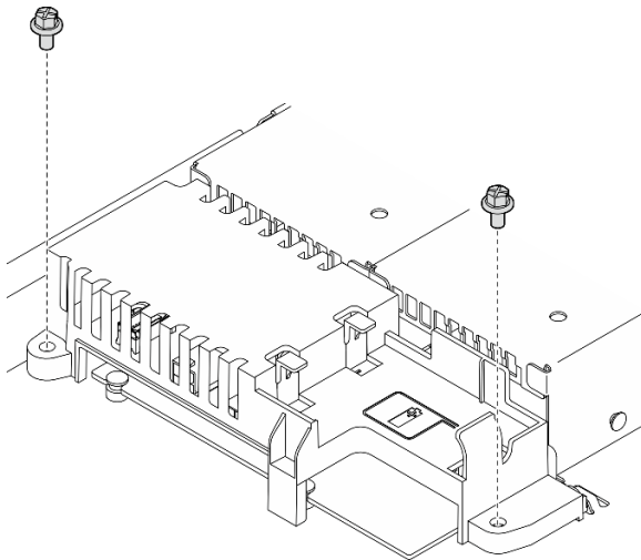
Figure 86. Retrait des vis du carter de PDB
