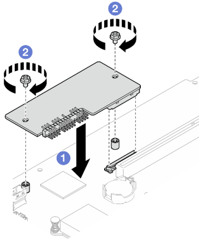
Figure 109. Installation du module de microprogramme et de sécurité RoT
