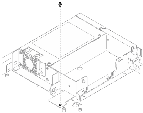
Figure 73. Retrait de la vis du support du bloc d'alimentation
