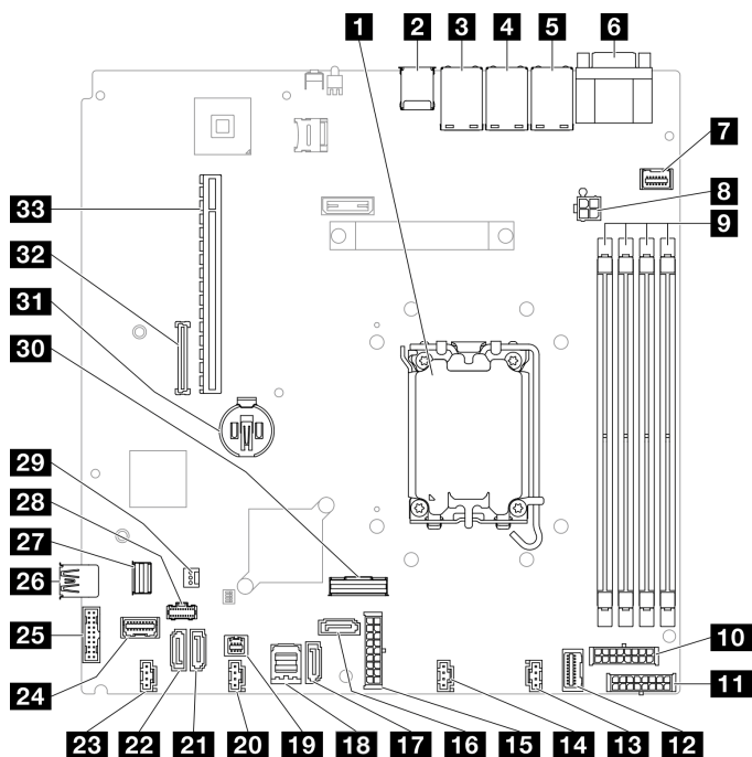
Figure 151. Connecteurs de la carte mère
