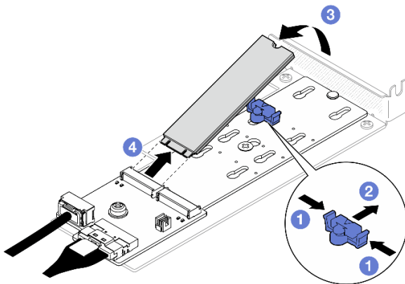
Figure 50. Retrait d'une unité M.2
