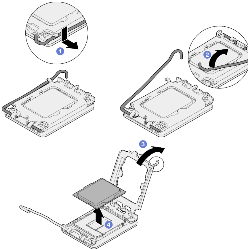
Figure 94. Ouverture du dispositif de retenue du processeur
