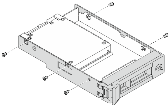
Figure 6. Retrait des vis de l'adaptateur d'unité
