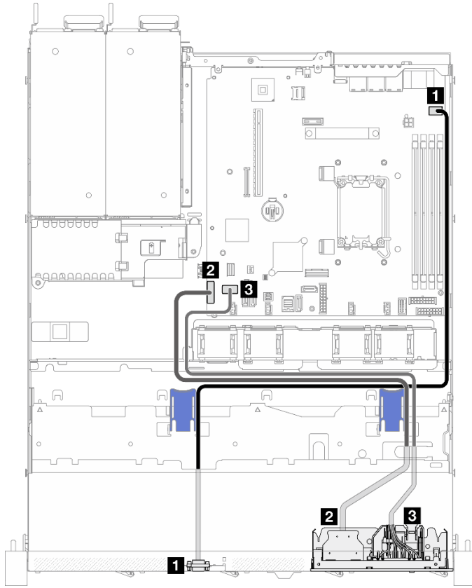
Figure 129. Cheminement des câbles du module d'E-S avant pour modèle 3,5 pouces
