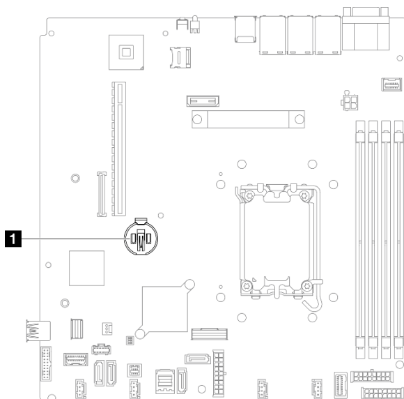
Figure 22. Emplacement de la pile CMOS
