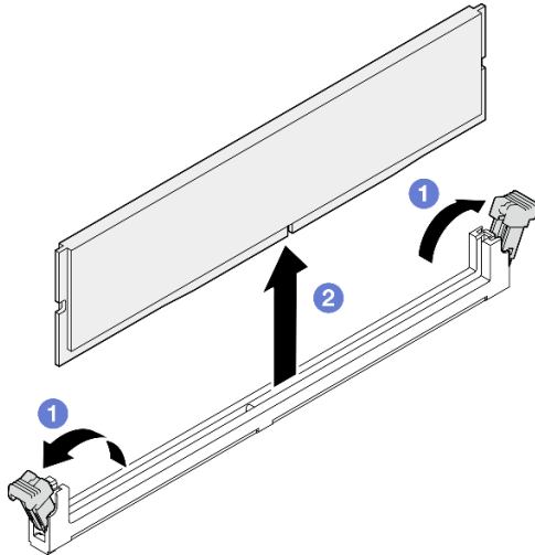
Figure 62. Retrait d'un module de mémoire
