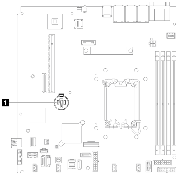
Figure 20. Emplacement de la pile CMOS
