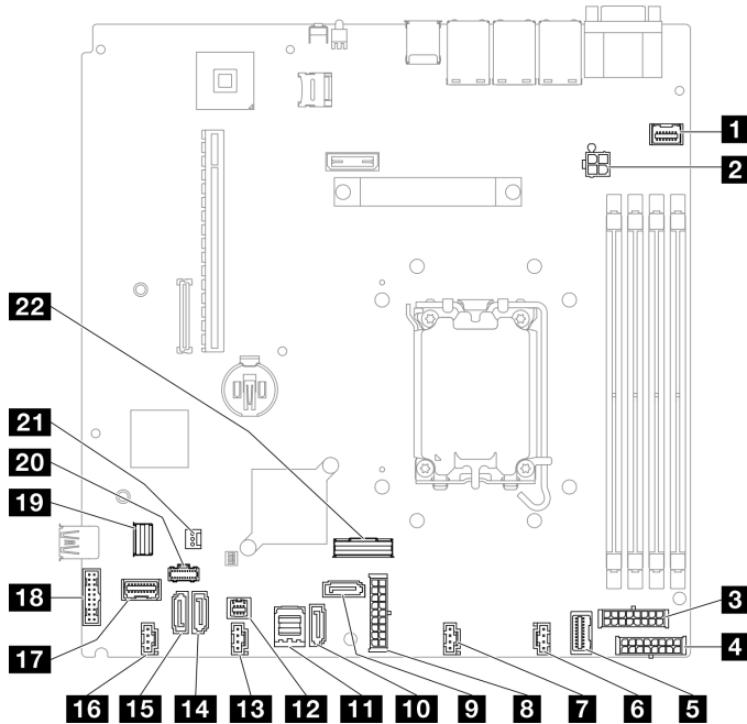
Figure 128. Connecteurs de la carte mère
