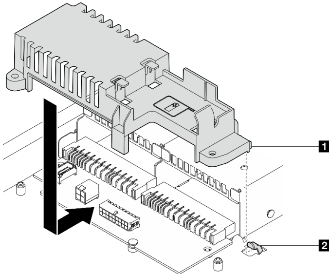
Figure 92. Installation du carter du tableau de distribution
