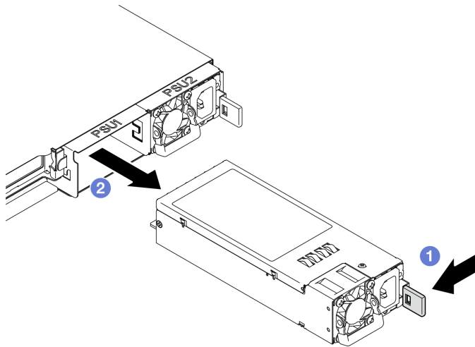
Figure 83. Unité de bloc d'alimentation remplaçable à chaud
