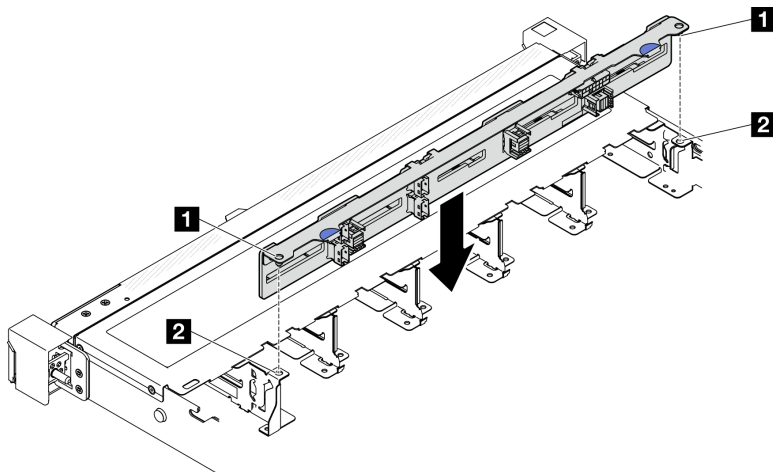
Figure 4. Installation de dix fonds de panier d'unité remplaçable à chaud 2,5 pouces
