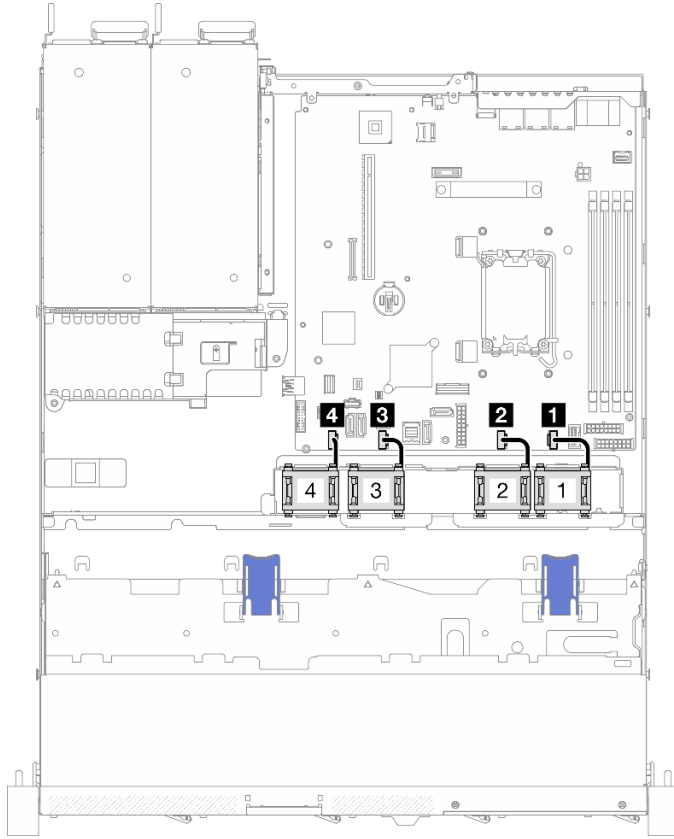
Figure 131. Cheminement des câbles de ventilateur
