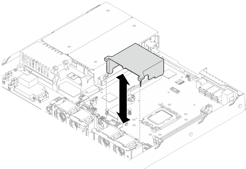
Figure 14. Retrait de la grille d'aération
