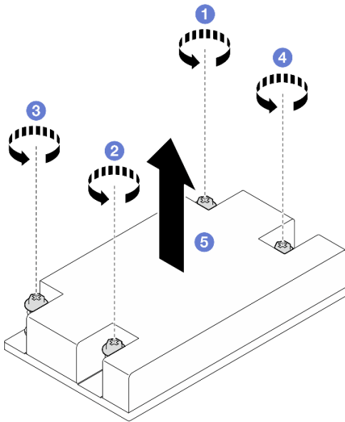
Figure 42. Retrait du dissipateur thermique
