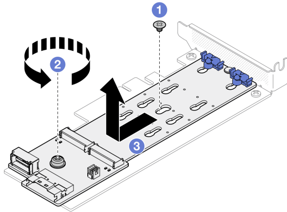
Figure 53. Retrait de l'adaptateur d'amorçage M.2
