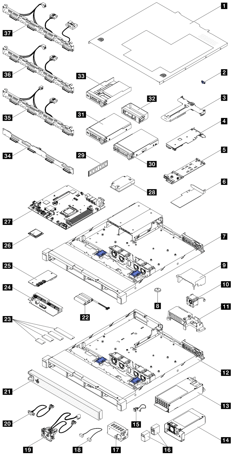
図 32. サーバー・コンポーネント - 3.5 型ドライブ・モデル
