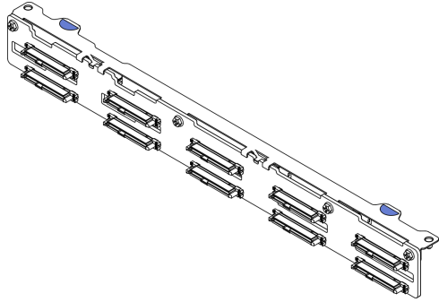
図 17. バックプレーン、10 個の 2.5 型ホット・スワップ・ドライブ
