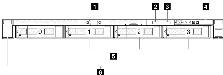
図 3. 3.5 型ホット・スワップ・ドライブ・モデルの前面図
