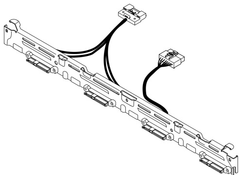
図 13. バックプレート、4台の3.5型シンプル・スワップ・ドライブ (Gen 4 RAID アダプターに接続)
