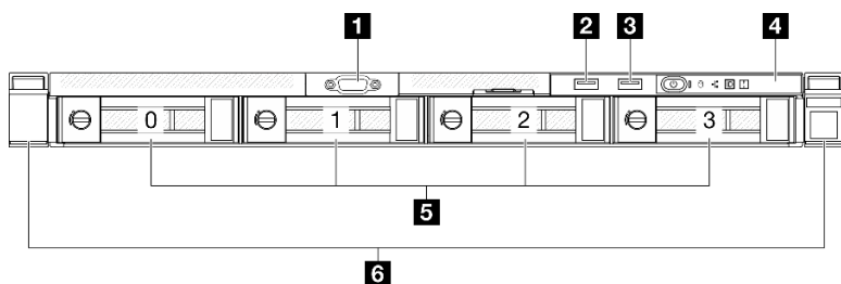
図 2. 3.5 型シンプル・スワップ・ドライブ・モデルの前面図
