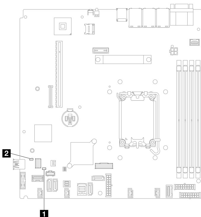
図 28. システム・ボード LED
