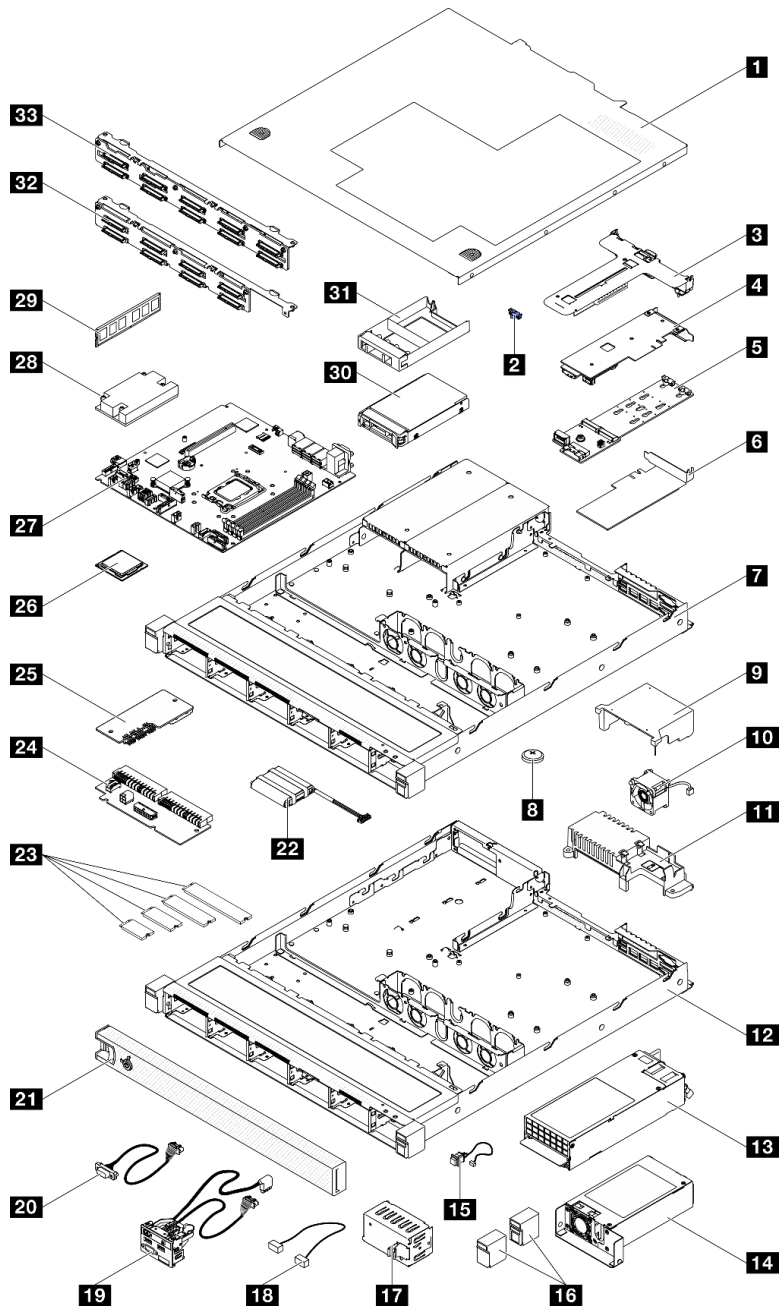
図 31. サーバー・コンポーネント - 2.5 型ドライブ・モデル
