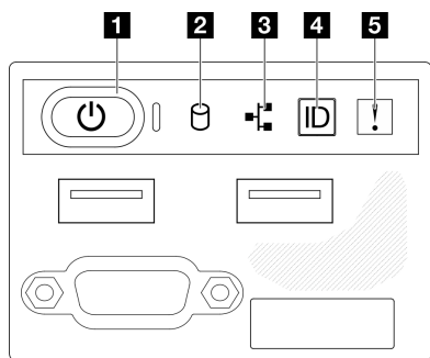
図9. 2.5 型ドライブ・シャーシの前面 I/O モジュール
