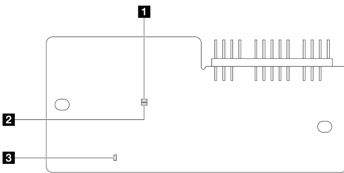
図 29. ファームウェアおよび RoT セキュリティー・モジュール 上の LED
