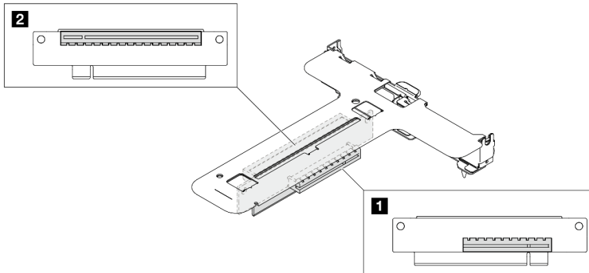
図 19. x16/x8 PCIe ライザー
