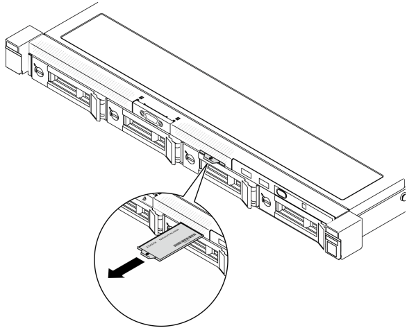
図 34. 引き出し式情報タブにあるLenovo XClarity Controller のネットワーク・アクセス・ラベル
