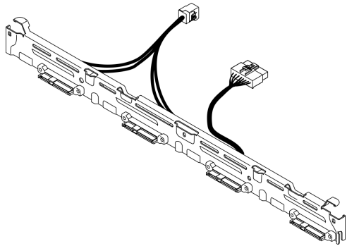
図 12. バックプレート、4台の3.5型シンプル・スワップ・ドライブ (Gen 3 RAID アダプターに接続)
