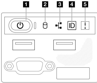
図 23. 2.5 型ドライブ・シャーシの前面 I/O モジュール
