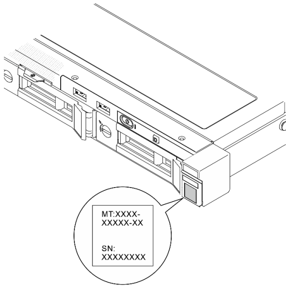
図 33. ID ラベルの位置
