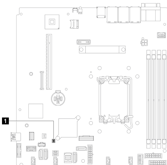
図21. システム・ボードのスイッチ
