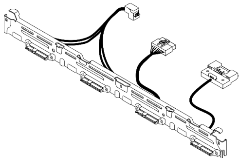
図 14. バックプレート、2台の3.5型シンプル・スワップ SATA ドライブおよび2台の NVMe ドライブ (オンボード・コネクタに接続)
