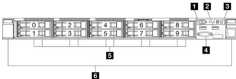
図4. 2.5 型ホット・スワップ・ドライブ・モデルの前面図
