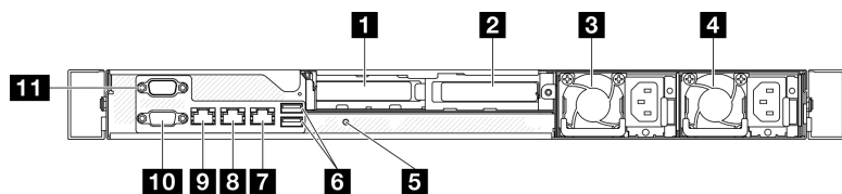
図6. ホット・スワップ・パワー・サプライ・モデルの背面図
