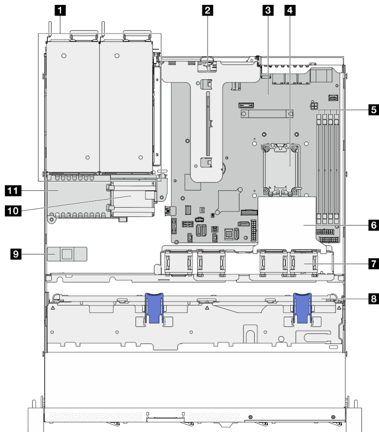
図8. サーバーの上部図 (3.5 型ドライブ・モデル)
