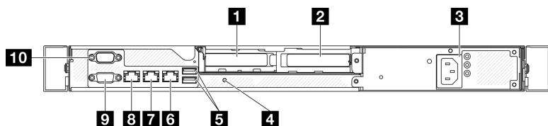
図 5. 固定パワー・サプライ・モデルの背面図
