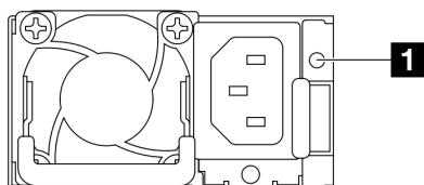
図 27. ホット・スワップ・パワー・サプライ・ユニット LED
