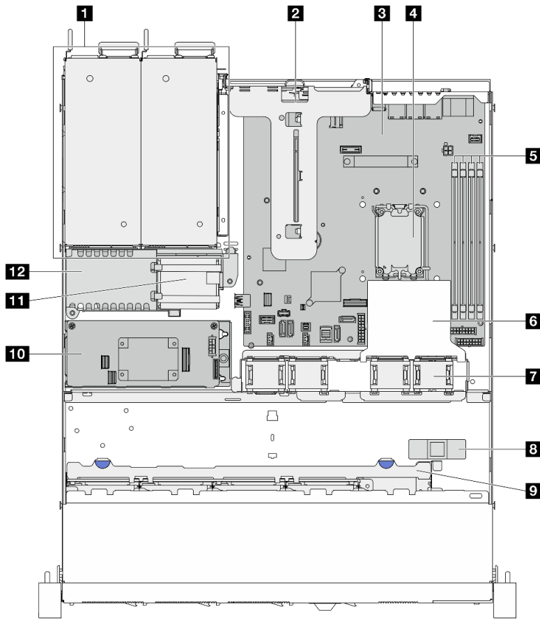
図7. サーバーの上部図 (2.5 型ドライブ・モデル)
