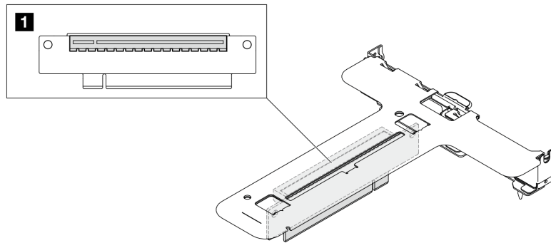
図 18. x16 PCIe ライザー
