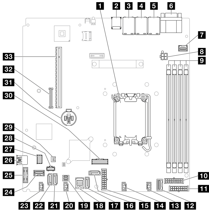
図 20. システム・ボード・コネクタ
