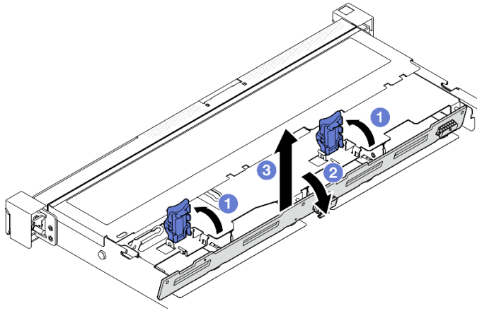
그림 12. 백플레이트 제거
