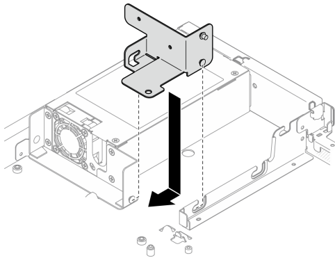
그림 81. 전원 공급 장치 브래킷 설치
