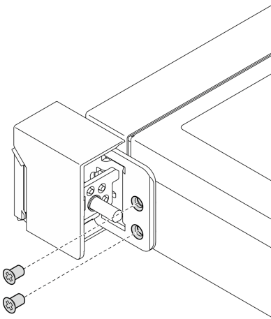
그림 102. 랙 래치 설치
