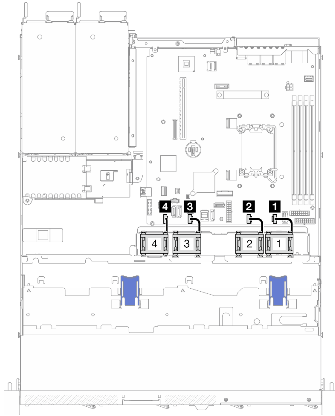
그림 131. 팬 케이블 배선
