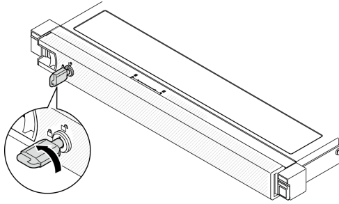
그림 107. 보안 베젤 잠금
