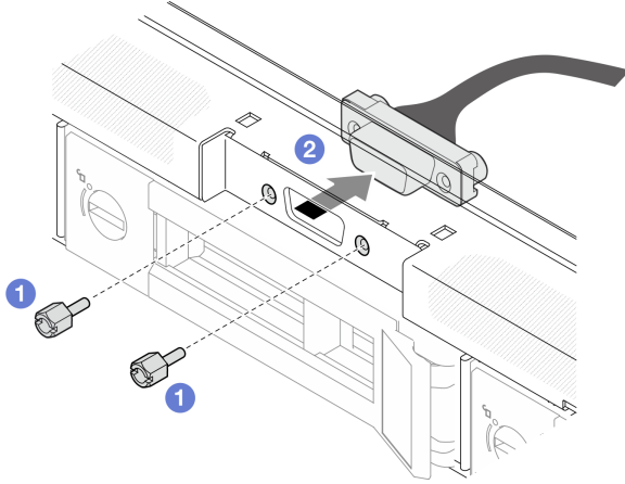
그림 119. VGA 케이블 제거
