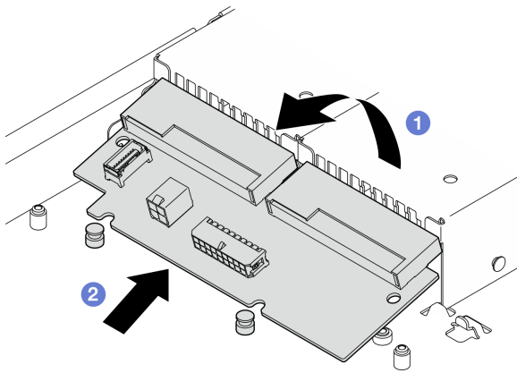
그림 89. 전원 분배 보드 제거
