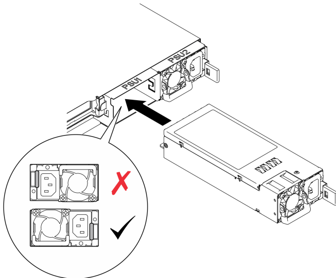
그림 85. 핫 스왑 전원 공급 장치 설치
