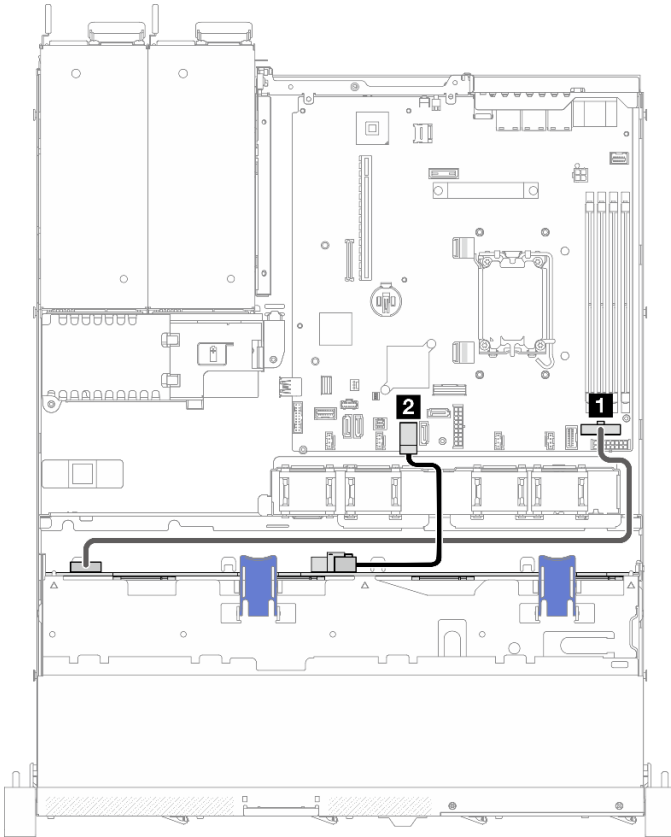
그림 142. 4개의 SATA/SAS 드라이브(소프트웨어 RAID)
