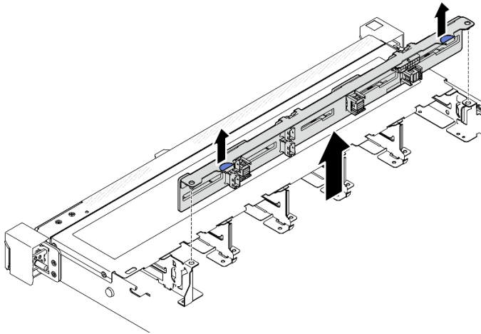
그림 2. 2.5인치 핫 스왑 드라이브 백플레인 10개 제거
