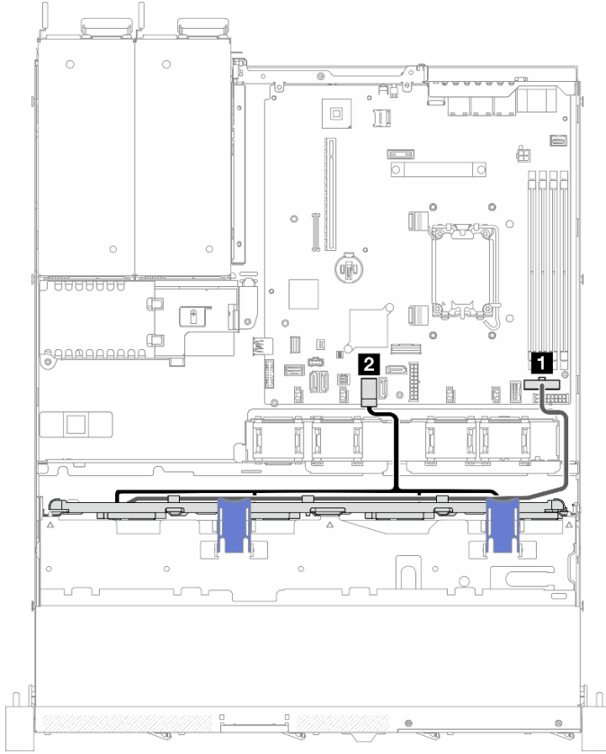
그림 139. 4개의 SATA 드라이브(소프트웨어 RAID)
