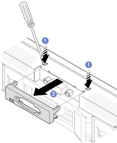
그림 118. VGA 덮개 제거
