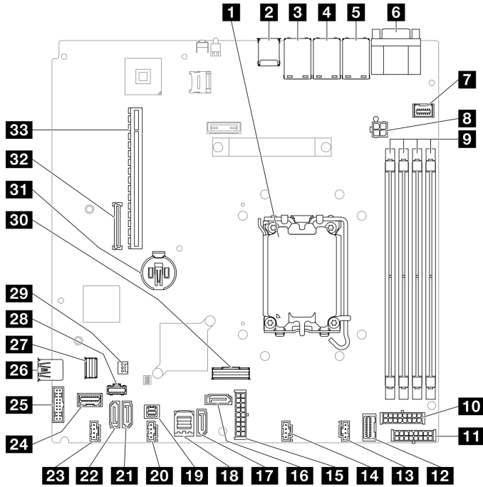
그림 151. 시스템 보드 커넥터
