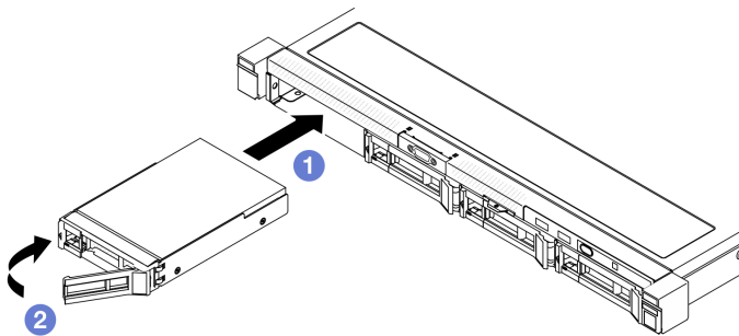
그림 29. 3.5인치 핫 스왑 드라이브 설치
