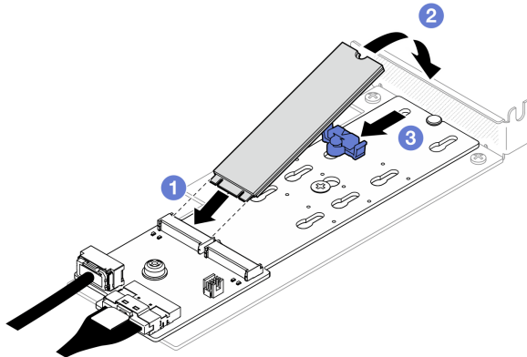
그림 60. M.2 드라이브 설치
