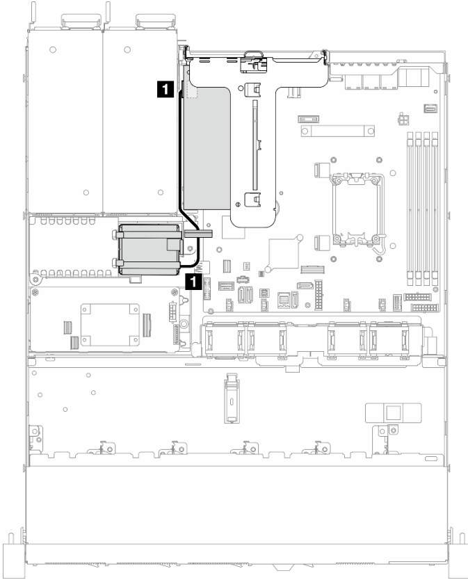
그림 134. 플래시 전원 모듈 케이블 배선
