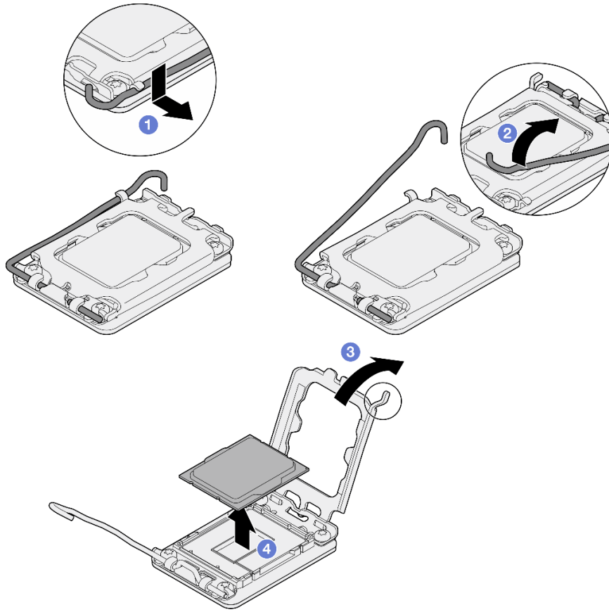
그림 94. 프로세서 고정장치 열기
