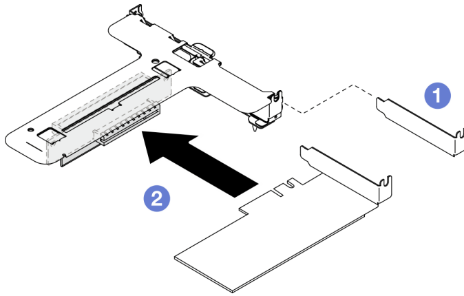
그림 69. PCIe 어댑터 설치(슬롯 1)
