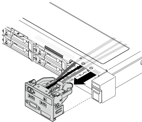
그림 35. 앞면 I/O 모듈 제거
