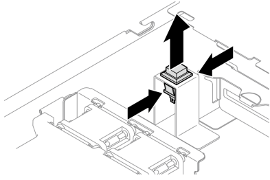
그림 46. 침입 스위치 제거
