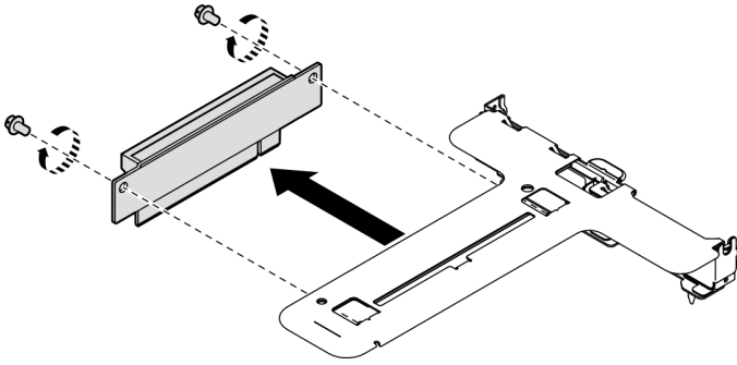
그림 66. PCIe 라이저 카드 제거
