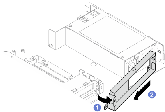
그림 76. 뒷면 브래킷 제거
