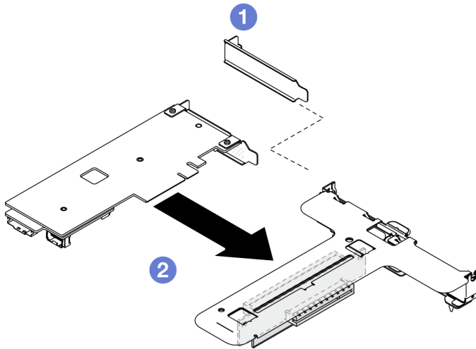
그림 70. PCIe 어댑터 설치(슬롯 2)
