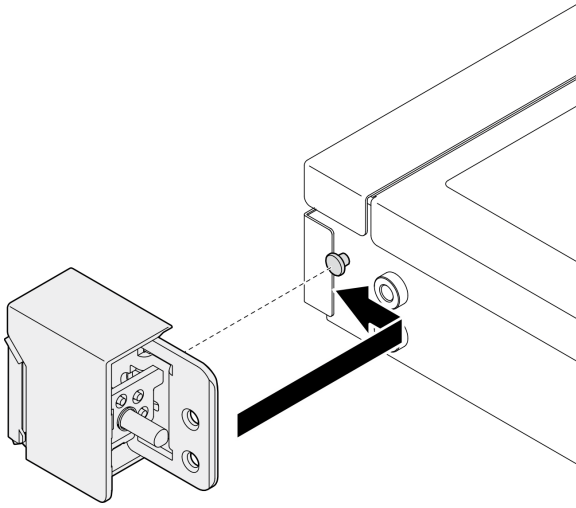
그림 101. 랙 래치 설치
