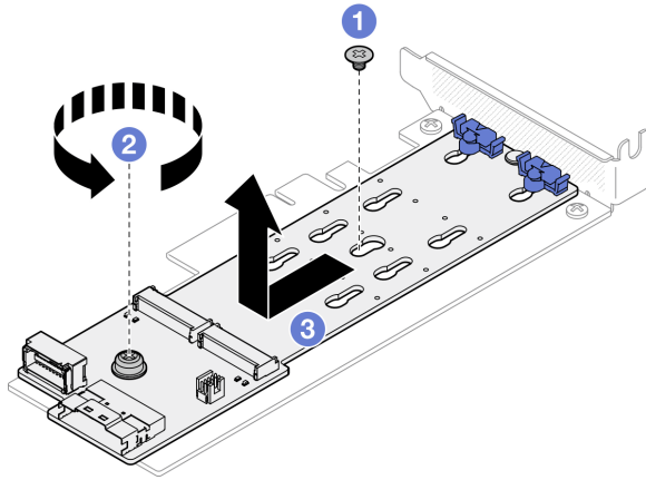
그림 53. M.2 부트 어댑터 제거
