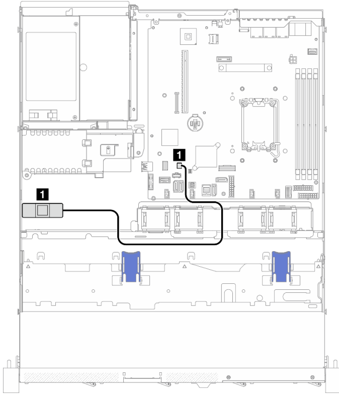
그림 135. 3.5인치 모델의 침입 스위치 케이블 배선
