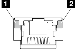
그림 160. XCC 시스템 관리 포트 LED
