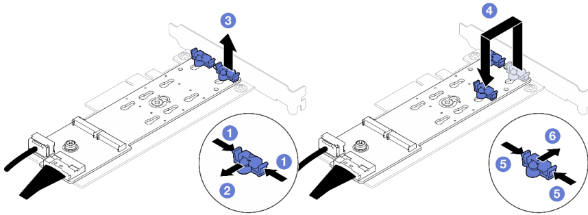
그림 54. M.2 고정장치 조정
