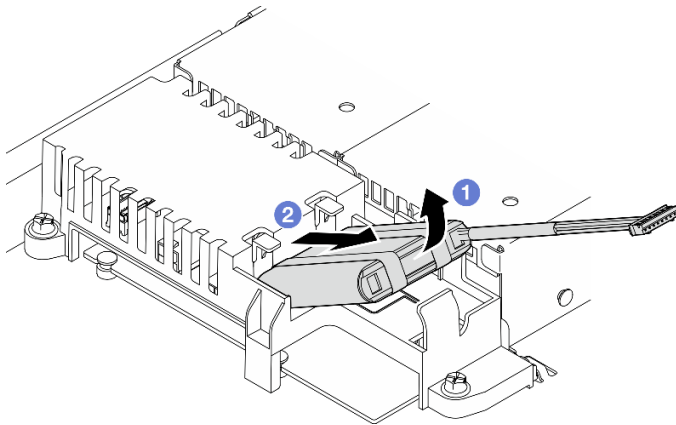
그림 32. 플래시 전원 모듈 제거
