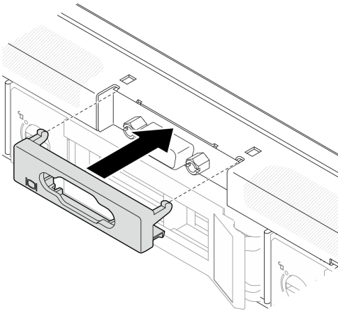
그림 121. VGA 덮개 설치
