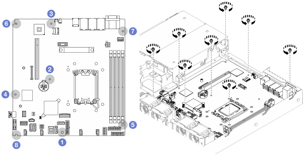
그림 110. 시스템 보드 나사 위치
