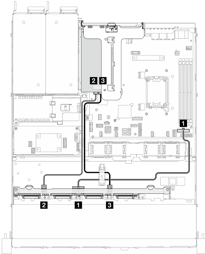
그림 145. 1개의 8i(하드웨어 RAID/HBA)가 포함된 8개의 SATA/SAS 드라이브
