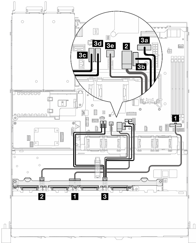
그림 144. 8개의 SATA/SAS 드라이브(소프트웨어 RAID)
