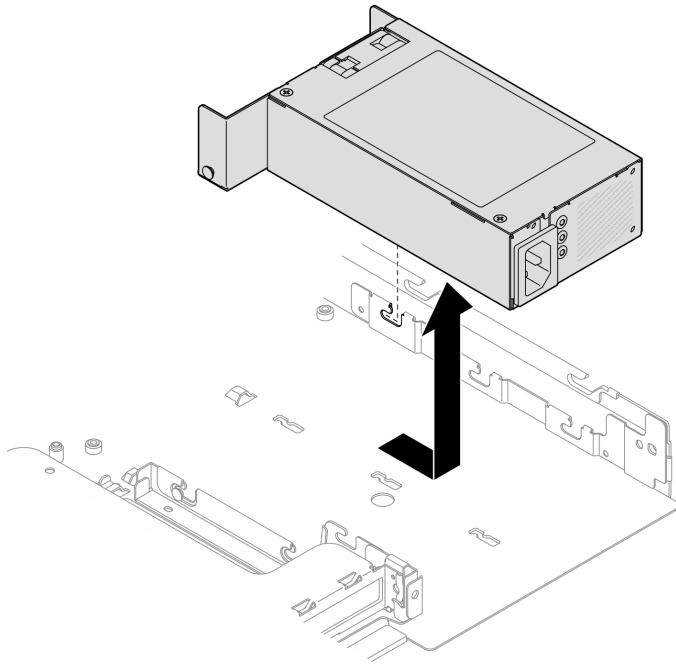
그림 77. 고정 전원 공급 장치 제거
