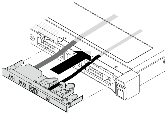
그림 40. 앞면 I/O 모듈 설치
