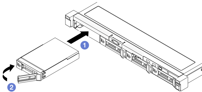
그림 25. 심플 스왑 드라이브 설치
