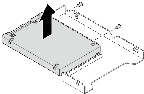
그림 7. 드라이브 어댑터에서 2.5인치 드라이브 제거
