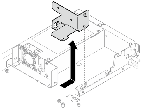
그림 74. 전원 공급 장치 브래킷 제거
