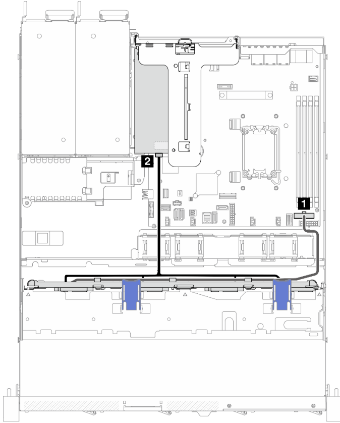
그림 141. 4개의 SATA 드라이브(하드웨어 RAID/HBA)
