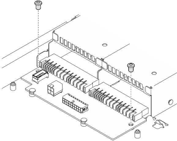
그림 88. 전원 분배 보드 나사 제거
