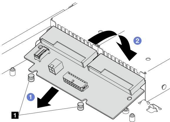
그림 90. 전원 분배 보드 설치
