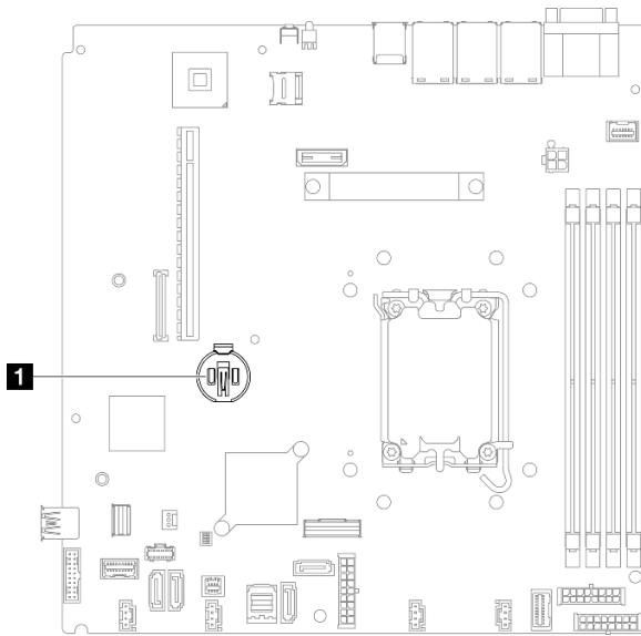
그림 22. CMOS 배터리 위치
