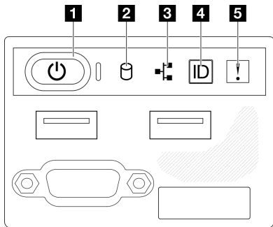
그림 153. 2.5인치 드라이브 새시 앞면 I/O 모듈
