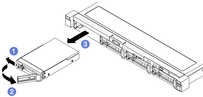
그림 27. 3.5인치 핫 스왑 드라이브 제거
