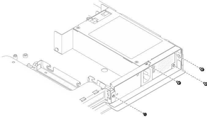
그림 75. 뒷면 브래킷 나사 제거
