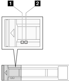
그림 152. 드라이브 LED
