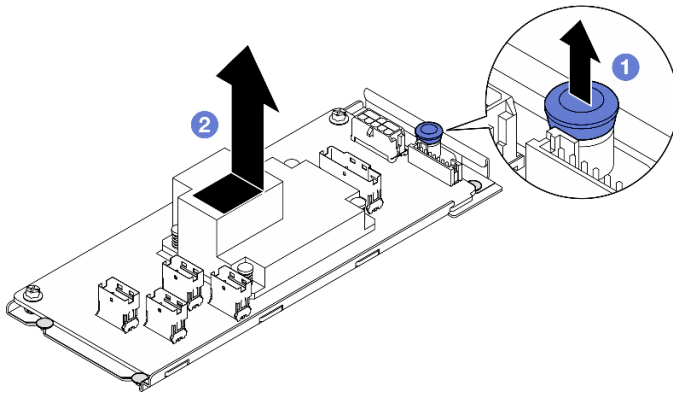
그림 16. 내부 CFF 어댑터 제거
