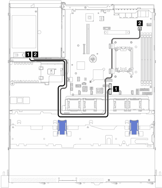
그림 132. 고정 전원 공급 장치 케이블 배선
