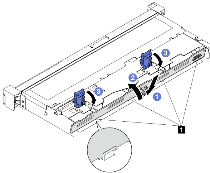
그림 13. 백플레이트 설치
