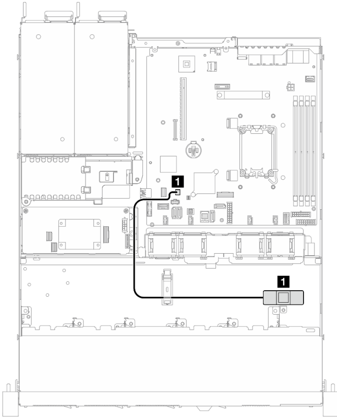
그림 136. 2.5인치 모델의 침입 스위치 케이블 배선
