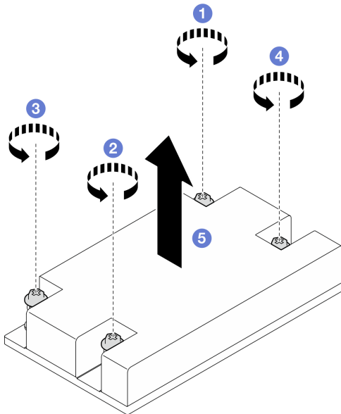
그림 42. 방열판 제거
