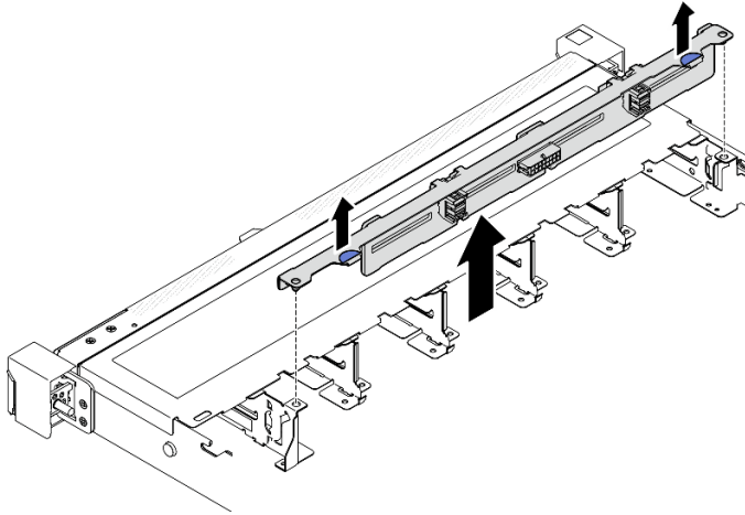
그림 3. 2.5인치 핫 스왑 드라이브 백플레인 8개 제거
