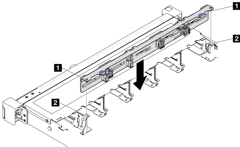
그림 4. 10개의 2.5인치 핫 스왑 드라이브 백플레인 설치
