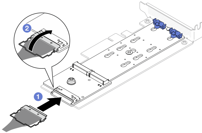
그림 58. SATA/NVMe M.2 부트 어댑터에 케이블 연결
