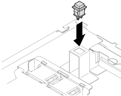
그림 49. 침입 스위치 설치
