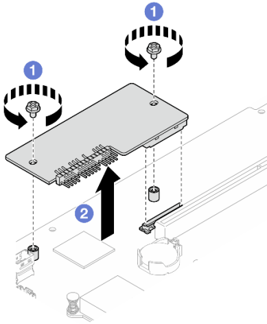
그림 108. 펌웨어 및 RoT 보안 모듈 제거
