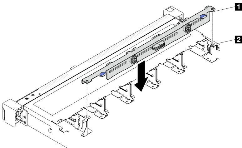
그림 5. 8개의 2.5인치 핫 스왑 드라이브 백플레인 설치
