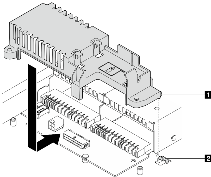
그림 92. 전원 분배 보드 덮개 설치
