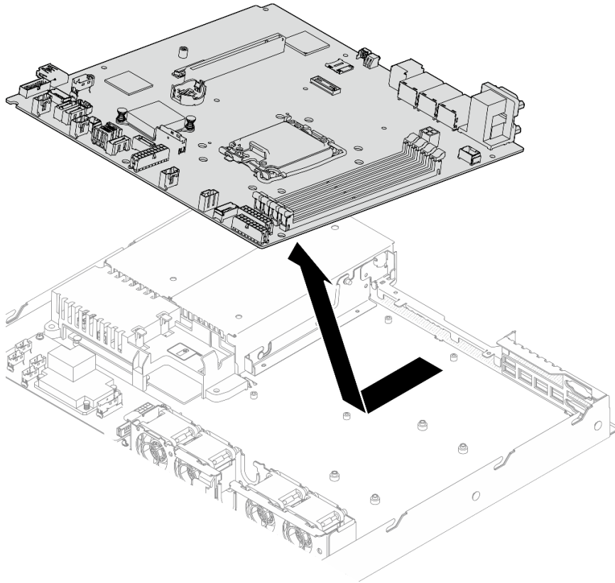
그림 111. 시스템 보드 제거
