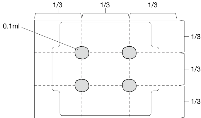
그림 97. 열 그리스의 적절한 형태
