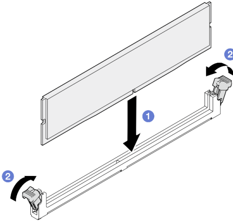
그림 64. 메모리 모듈 설치
