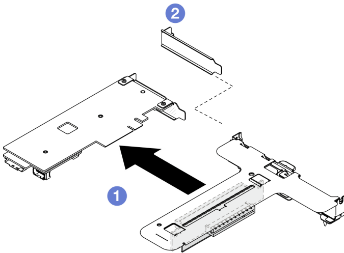
그림 68. PCIe 어댑터 제거(슬롯 2)
