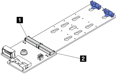
그림 59. M.2 드라이브 슬롯
