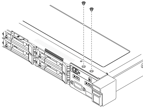
그림 37. 나사 설치
