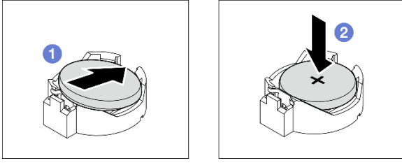
그림 23. CMOS 배터리 설치
