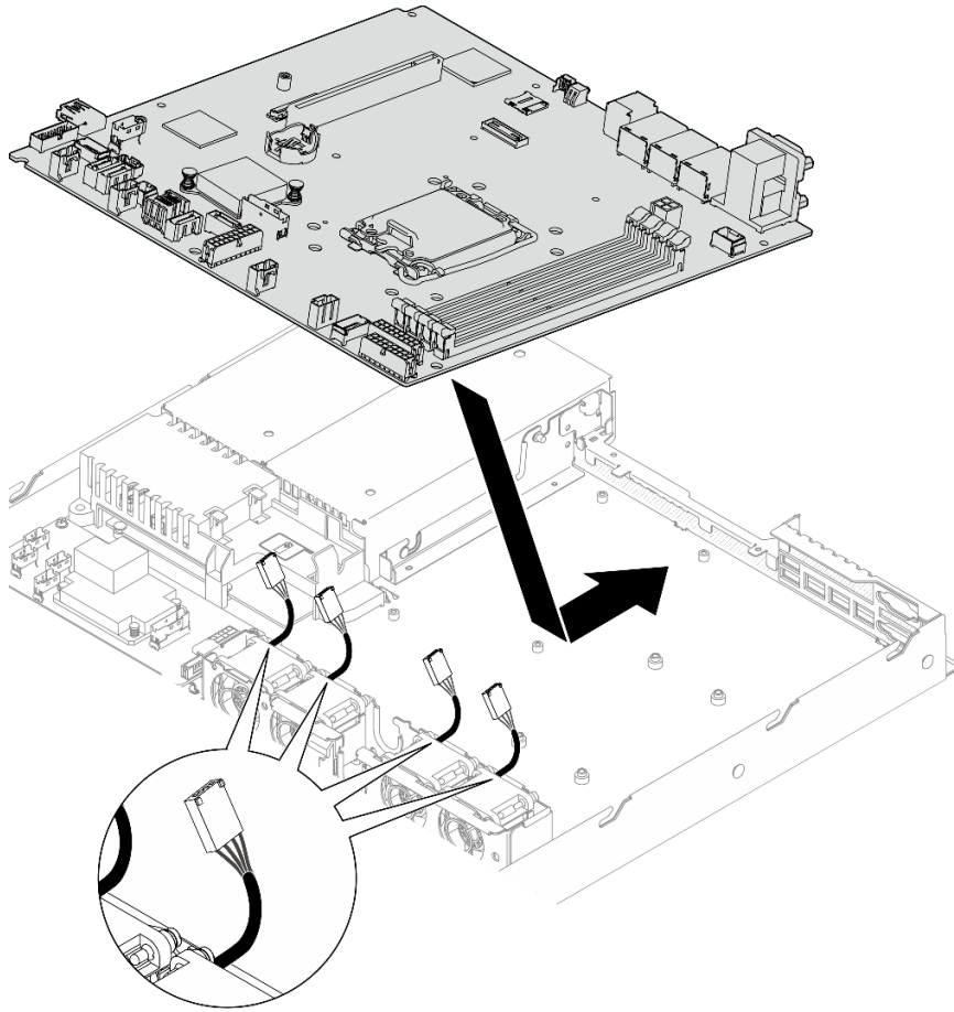
그림 112. 시스템 보드 설치
