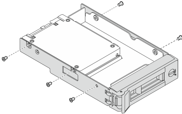
그림 6. 드라이브 어댑터에서 나사 제거
