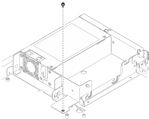
그림 82. 전원 공급 장치 브래킷 나사 설치
