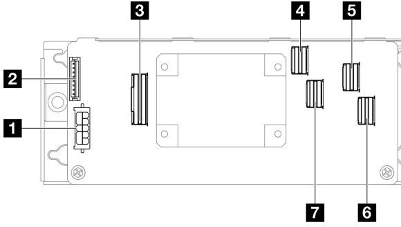
그림 123. CFF 16i RAID 어댑터 커넥터
