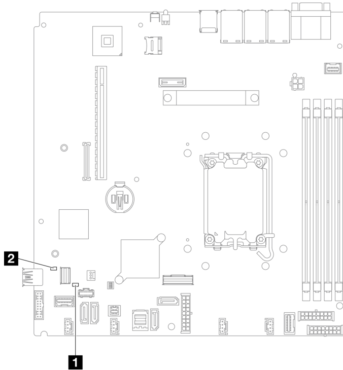
그림 158. 시스템 보드 LED
