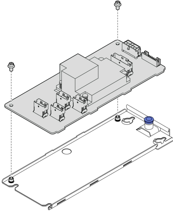
그림 17. 내부 CFF 어댑터 트레이 제거
