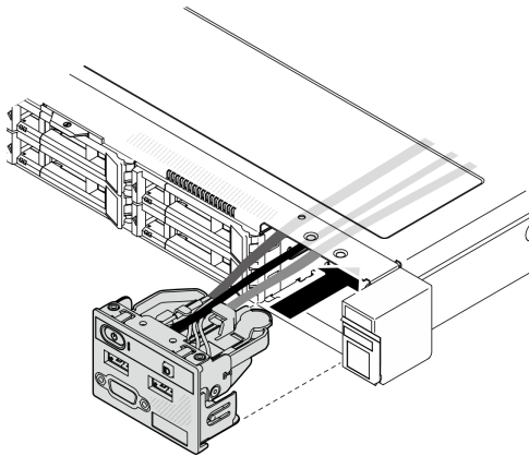
그림 36. 앞면 I/O 모듈(2.5인치 드라이브 모델) 설치
