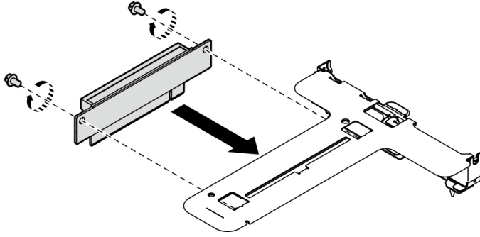
그림 71. PCIe 라이저 카드 설치
