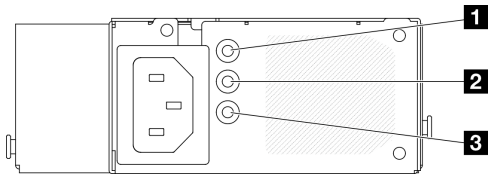
그림 156. 고정 전원 공급 장치 LED
