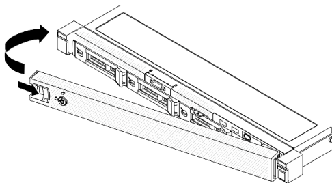
그림 106. 보안 베젤 설치
