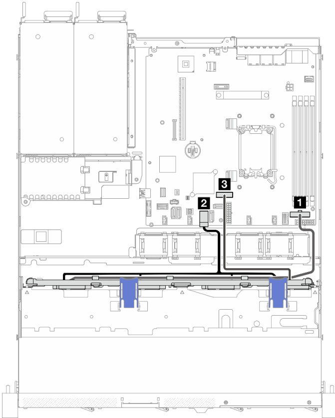
그림 140. SATA 드라이브 2개 및 NVMe 드라이브 2개(소프트웨어 RAID)
