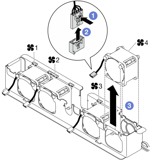
그림 30. 팬 제거
