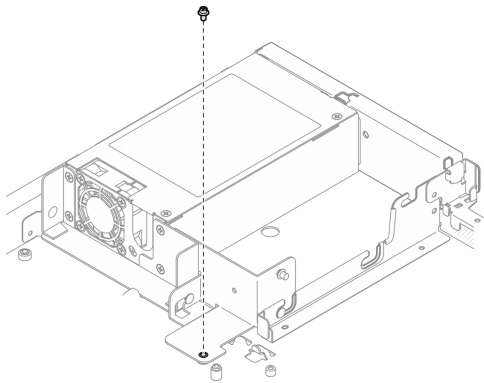
그림 73. 전원 공급 장치 브래킷 나사 제거
