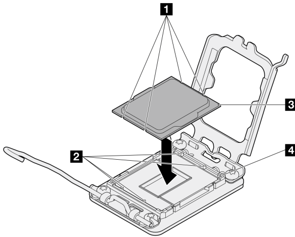
그림 95. 프로세서 설치
