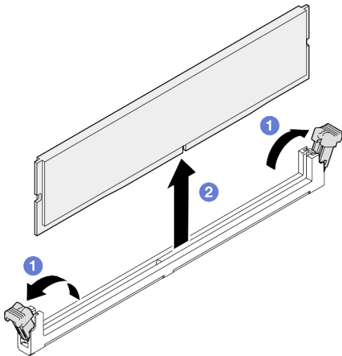
그림 62. 메모리 모듈 제거
