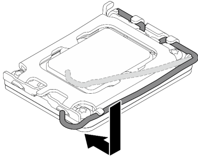
그림 96. 프로세서 고정장치 달기
