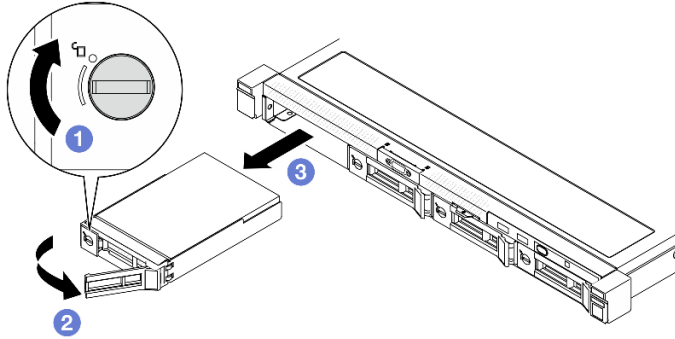
그림 24. 심플 스왑 드라이브 제거
