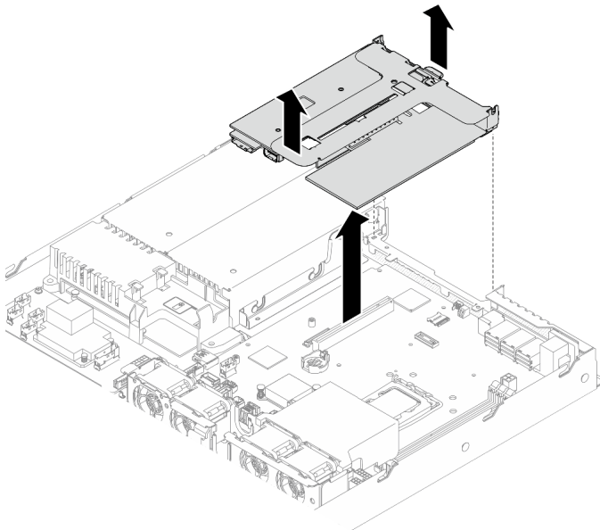
그림 65. PCIe 라이저 어셈블리 제거
