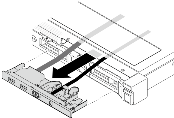
그림 39. 앞면 I/O 모듈 제거
