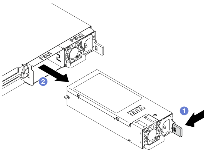
그림 83. 핫 스왑 전원 공급 장치
