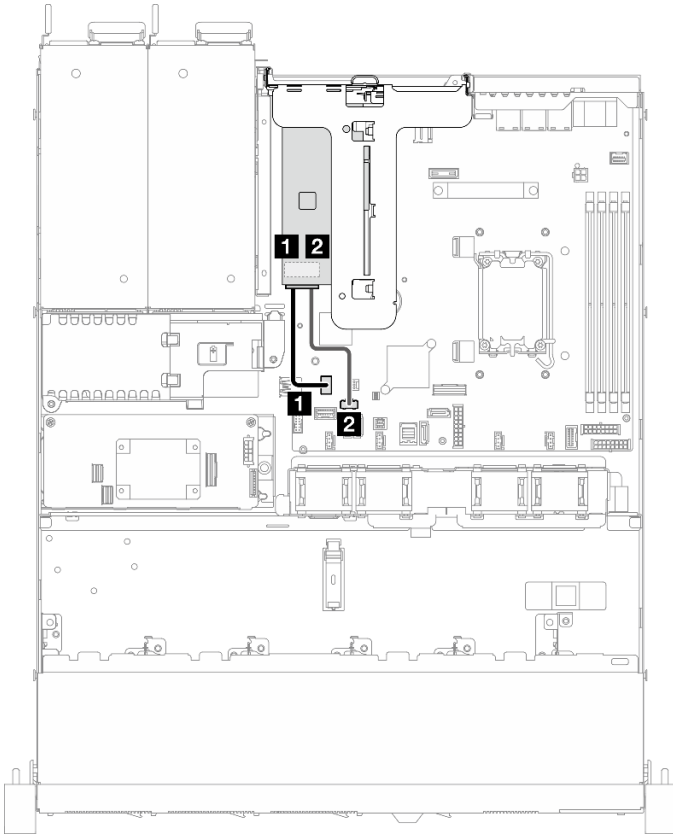
그림 138. SATA/NVMe M.2 부트 어댑터 케이블 배선
