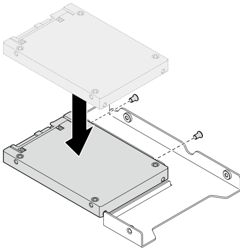
그림 8. 드라이브 어댑터에 2.5인치 드라이브 설치
