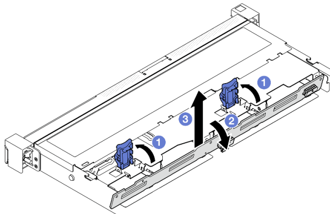
그림 10. 3.5인치 백플레인 제거
