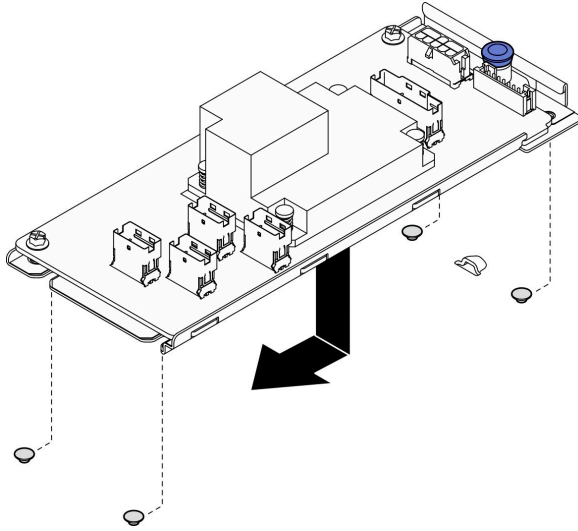
그림 19. 내부 CFF 어댑터 설치
