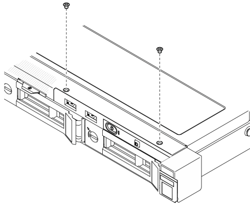
그림 41. 앞면 I/O 모듈 설치
