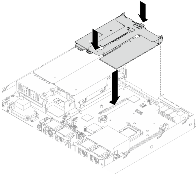
그림 72. PCIe 라이저 어셈블리 설치
