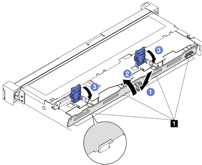
그림 11. 3.5인치 백플레인 설치
