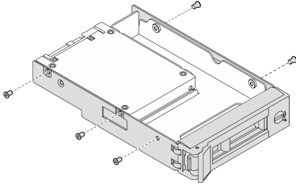
그림 9. 드라이브 어댑터에 나사 설치
