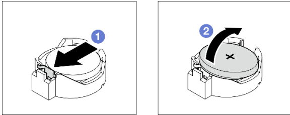
그림 21. CMOS 배터리 제거
