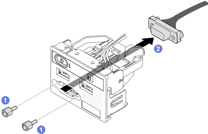
그림 116. VGA 케이블 제거
