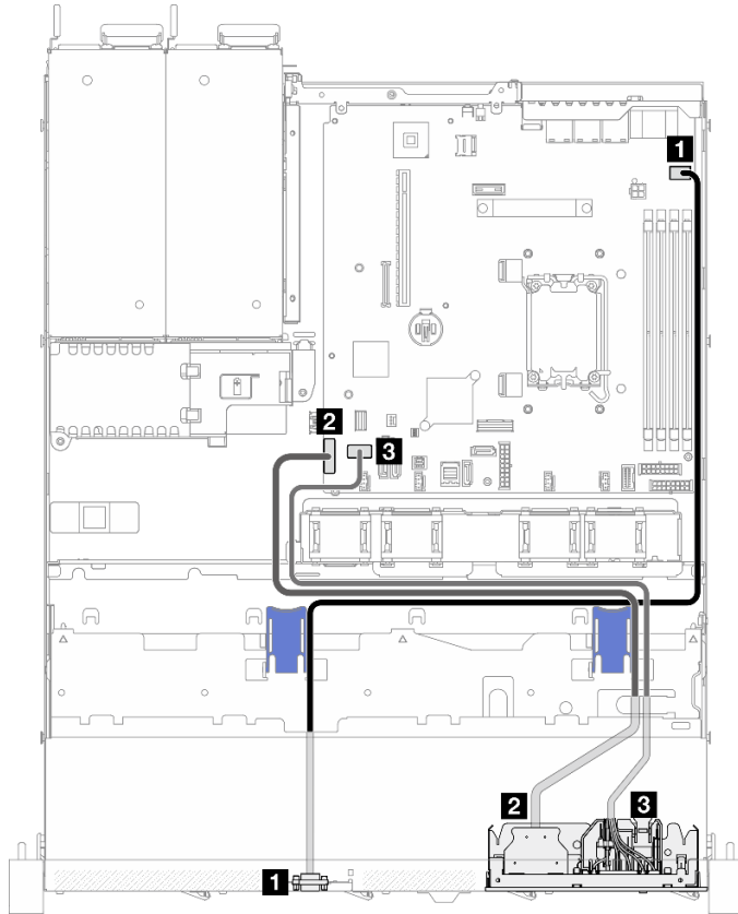
그림 129. 3.5인치 모델의 앞면 I/O 모듈 케이블 배선
