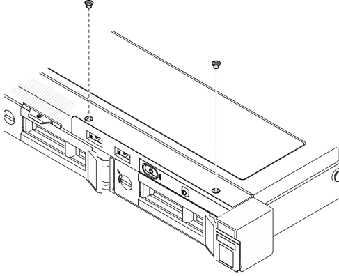
그림 38. 앞면 I/O 모듈 제거
