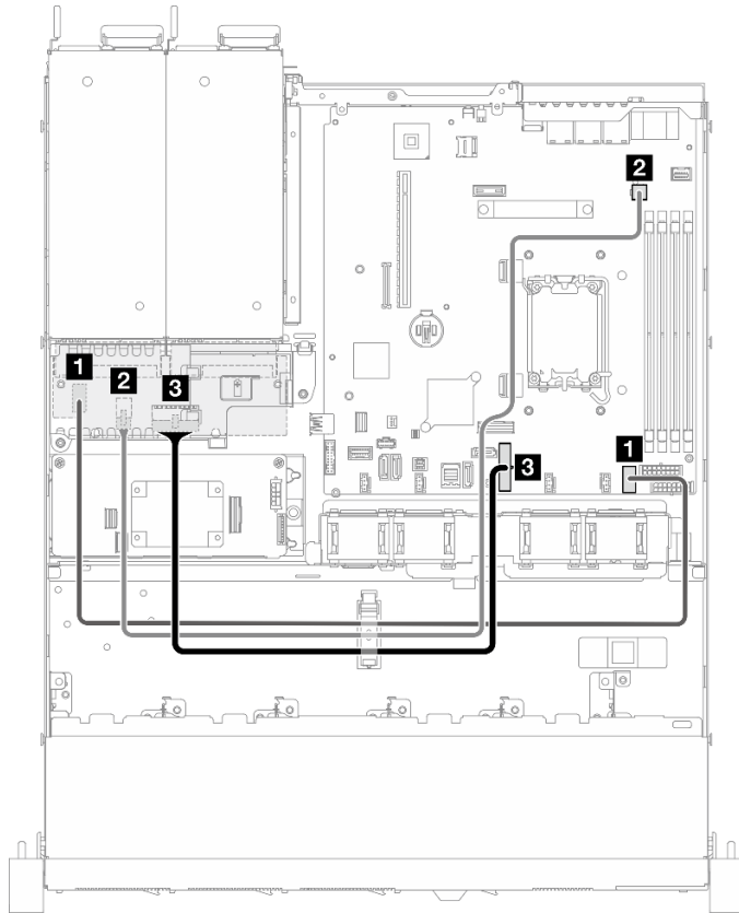
그림 133. 전원 분배 보드 케이블 배선
