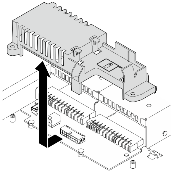
그림 87. 전원 분배 보드 덮개 제거
