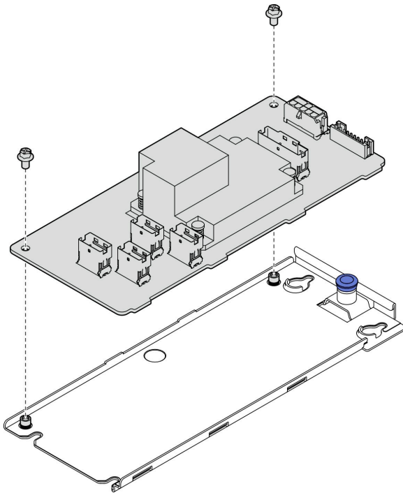
그림 18. 내부 CFF 어댑터 트레이 설치
