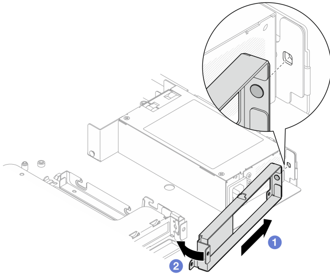
그림 79. 뒷면 브래킷 설치
