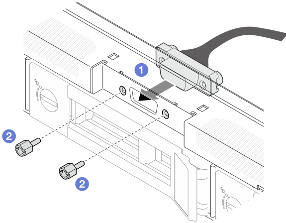
그림 120. VGA 케이블 설치
