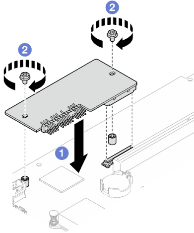
그림 109. 펌웨어 및 RoT 보안 모듈 설치
