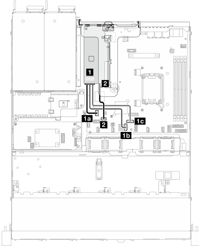
그림 137. SATA/x4 NVMe M.2 부트 어댑터 케이블 배선
