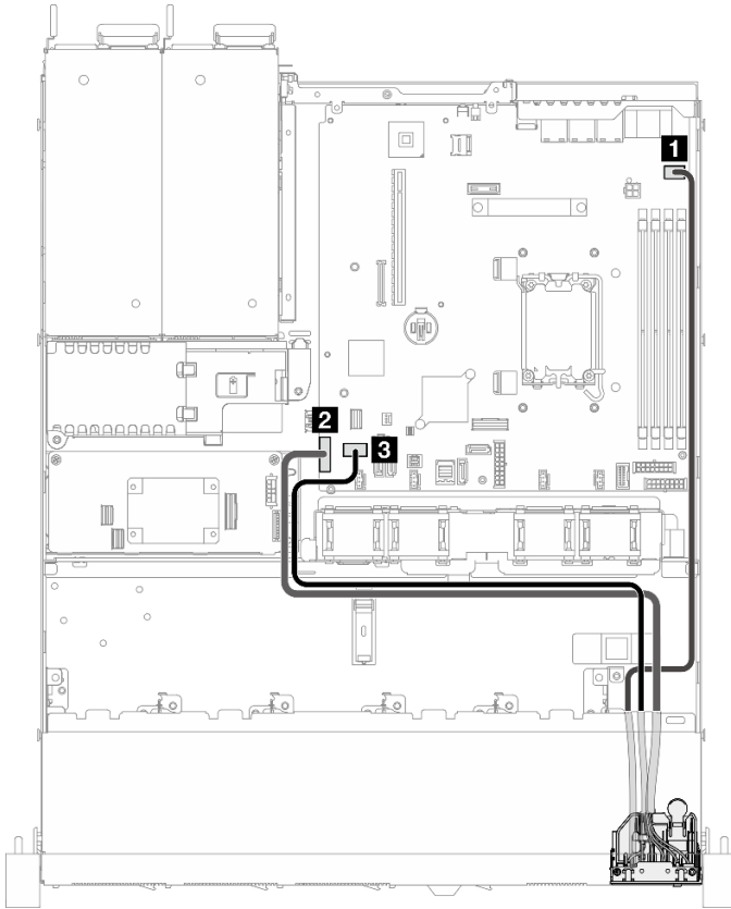
그림 130. 2.5인치 모델의 앞면 I/O 모듈 케이블 배선
