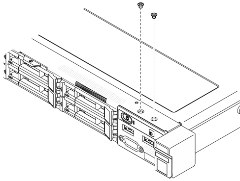
그림 34. 앞면 I/O 모듈 나사 제거
