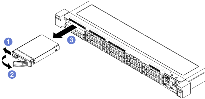
그림 26. 2.5인치 핫 스왑 드라이브 제거
