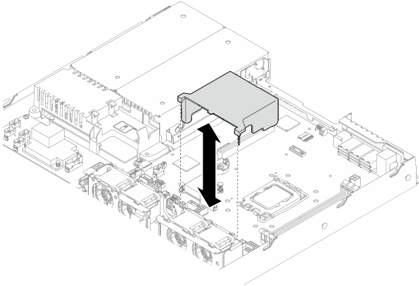
그림 15. 공기 조절 장치 설치
