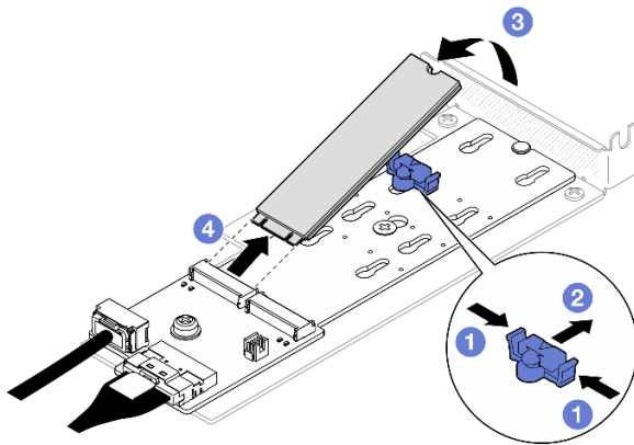
그림 50. M.2 드라이브 제거
