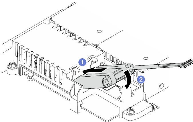
그림 33. 플래시 전원 모듈 설치
