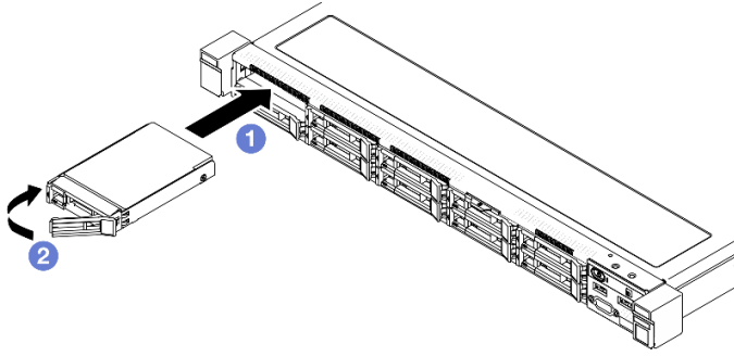
그림 28. 2.5인치 핫 스왑 드라이브 설치
