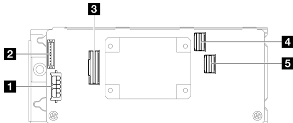
그림 122. CFF 8i RAID 어댑터 커넥터
