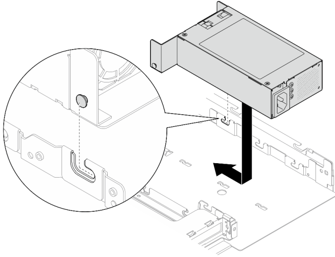
그림 78. 고정 전원 공급 장치 설치
