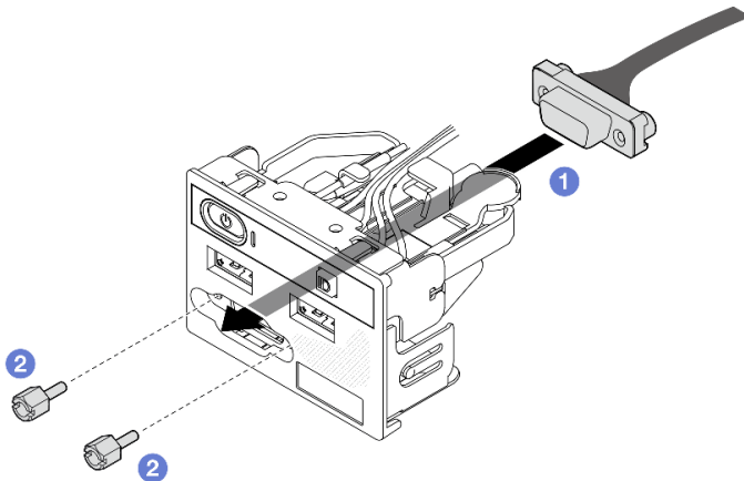
그림 117. VGA 케이블 설치
