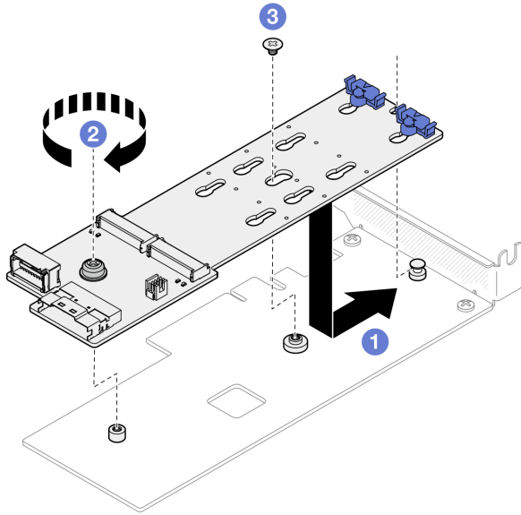
그림 56. M.2 부트 어댑터 설치
