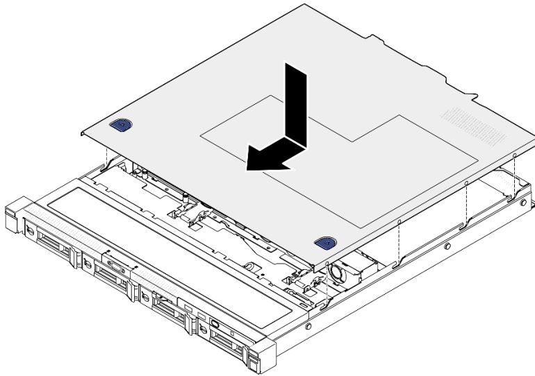
그림 115. 윗면 덮개 설치
