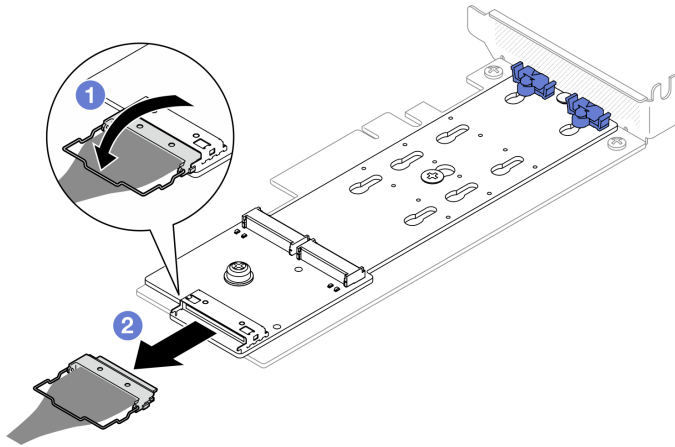
그림 52. SATA/NVMe M.2 부트 어댑터에서 케이블 분리
