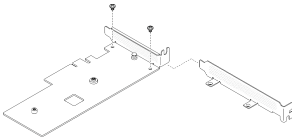
그림 55. 로우 프로파일 브래킷 설치
