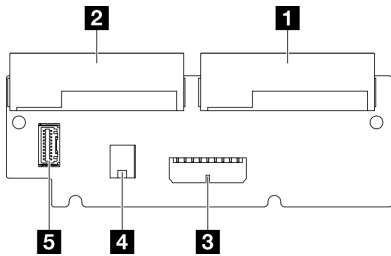
그림 127. 전원 분배 보드 커넥터
