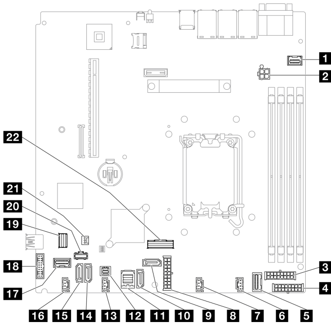
그림 128. 시스템 보드 커넥터
