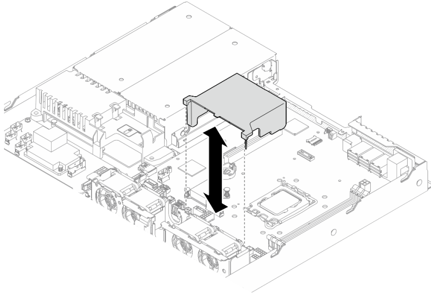
그림 14. 공기 조절 장치 제거
