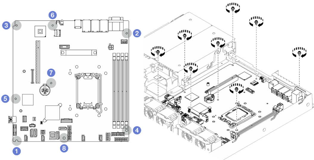
그림 113. 시스템 보드 나사 위치
