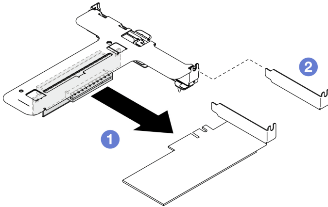
그림 67. PCIe 어댑터 제거(슬롯 1)
