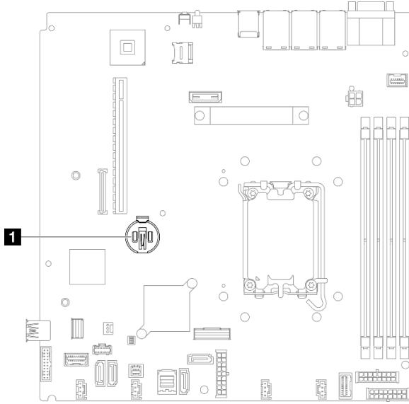
그림 20. CMOS 배터리 위치
