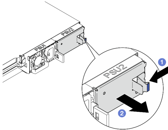
그림 84. PSU 필터 제거
