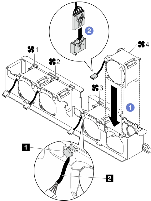
그림 31. 팬 설치
