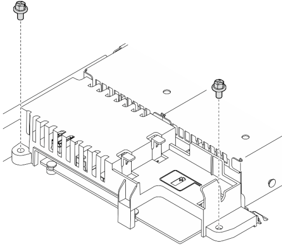
그림 93. PDB 덮개 나사 설치
