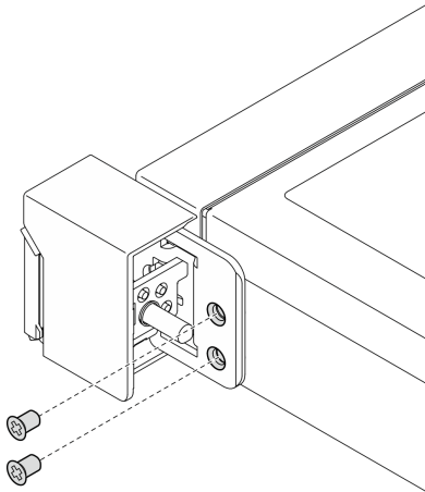
그림 99. 랙 래치 제거
