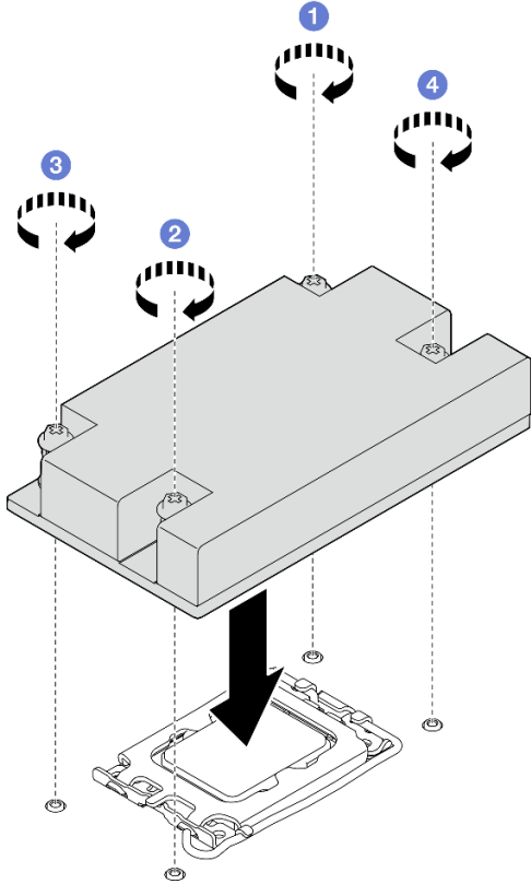
그림 43. 방열판 설치
