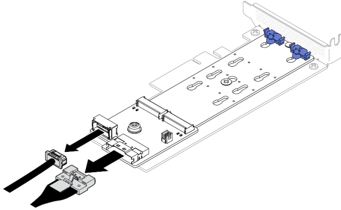
그림 51. SATA/x4 NVMe M.2 부트 어댑터에서 케이블 분리
