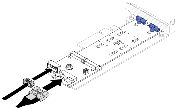
그림 57. SATA/x4 NVMe M.2 부트 어댑터에 케이블 연결
