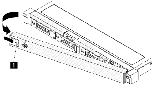
그림 105. 보안 베젤 제거
