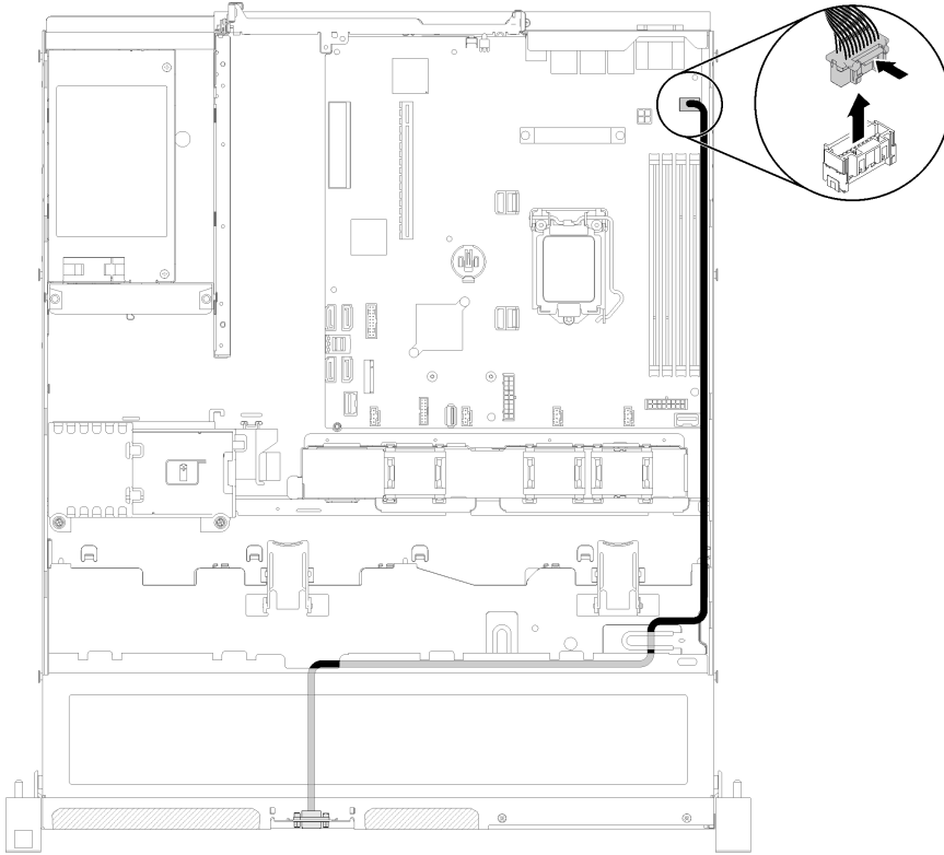
그림 131. VGA 케이블 제거 - 3.5인치 HDD 모델
