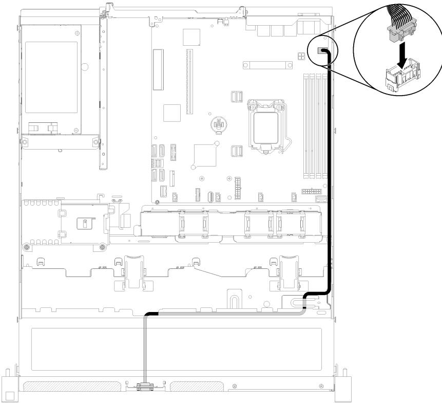
그림 135. VGA 케이블 설치
