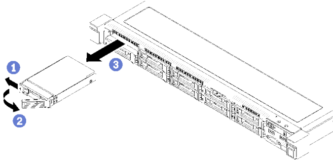
그림 59. 2.5인치 핫 스왑 드라이브 제거
