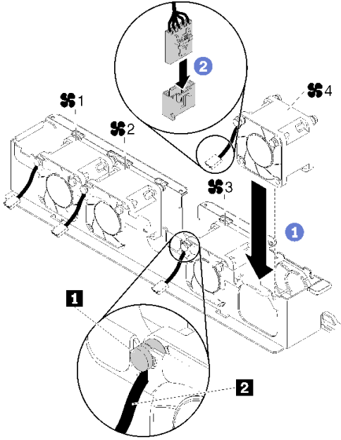
그림 64. 팬 설치
