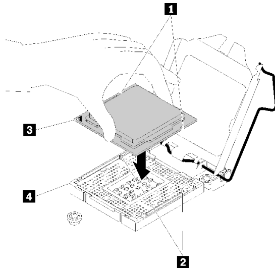
그림 107. 프로세서 설치
