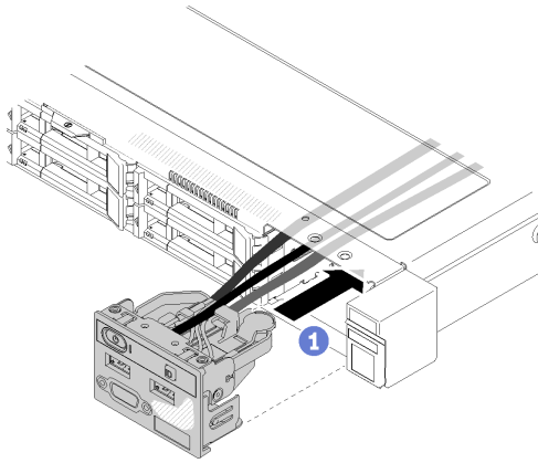
그림 71. 앞면 오퍼레이터 패널(2.5인치 HDD 모델) 설치
