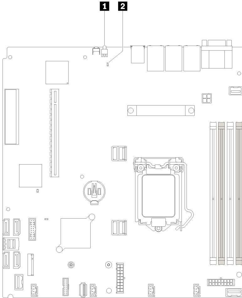
그림 13. 시스템 보드 LED
