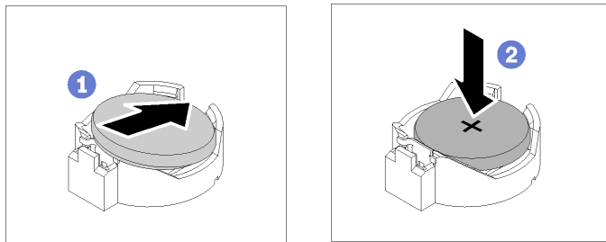
그림 52. CMOS 배터리 설치
