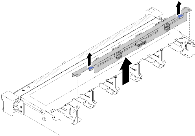
그림 46. 3.5인치 핫 스왑 드라이브 백플레인 제거
