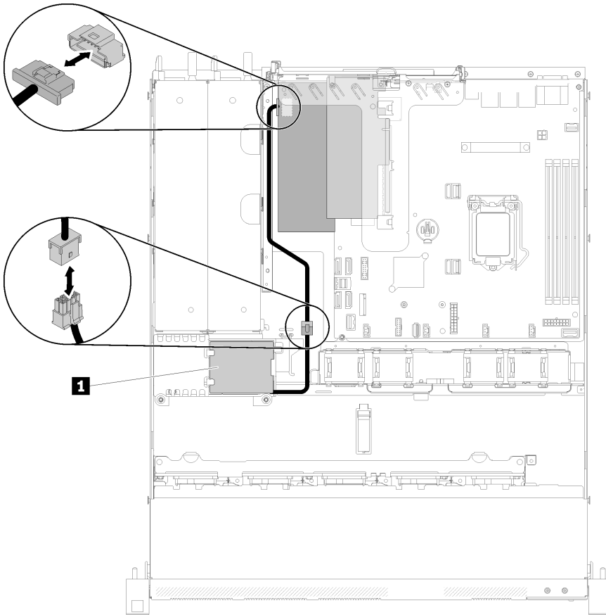
그림 96. 플래시 전원 모듈 케이블 분리
