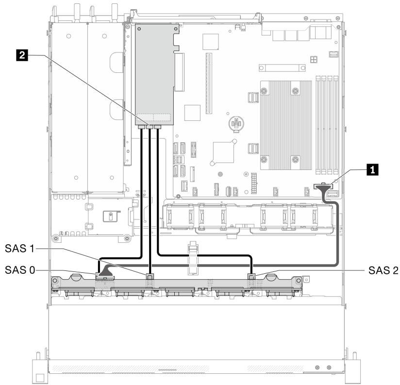
그림 37. 하드웨어 RAID가 있는 10개의 2.5인치 핫 스왑 드라이브 모델
