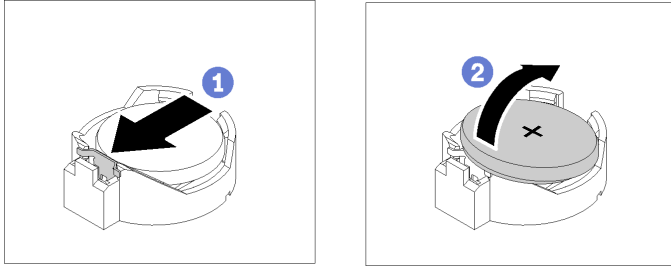
그림 51. CMOS 배터리 제거
