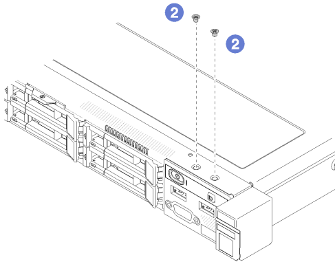
그림 72. 나사 설치
