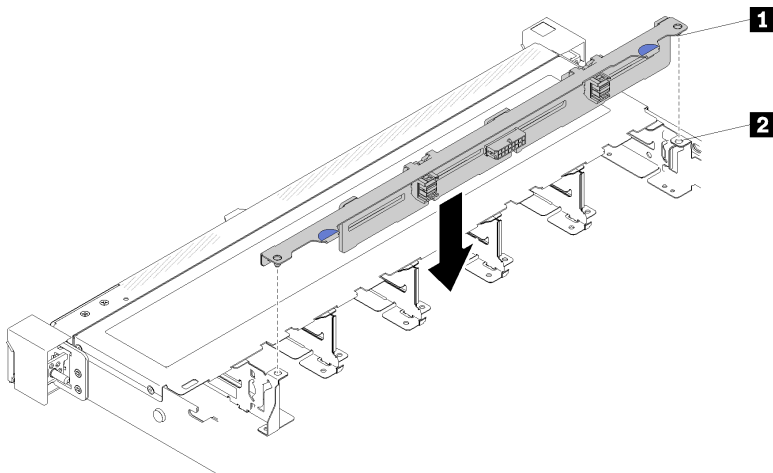
그림 48. 3.5인치 핫 스왑 드라이브 백플레인 설치
