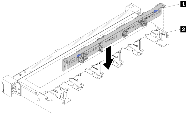
그림 47. 2.5인치 핫 스왑 드라이브 백플레인 설치
