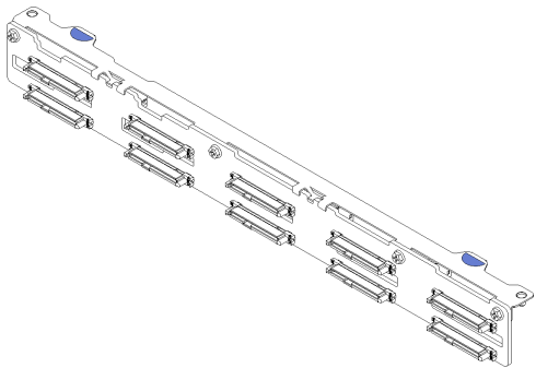
그림 22. 백플레인, 10개의 2.5인치 핫 스왑 드라이브
