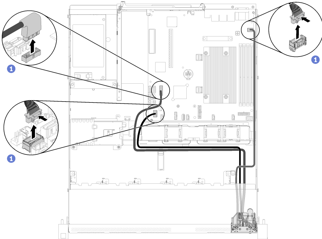
그림 68. 앞면 오퍼레이터 패널(2.5인치 HDD 모델) 케이블 제거
