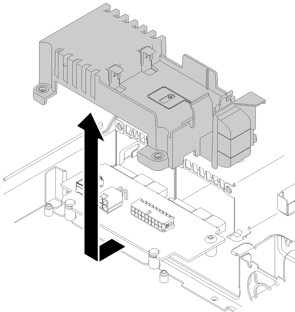
그림 98. 전원 인터페이스 보드 덮개 제거
