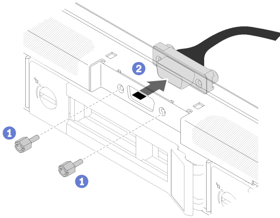
그림 133. VGA 케이블 제거
