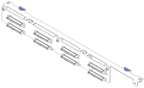
그림 21. 백플레인, 핫 스왑 2.5인치 드라이브 8개
