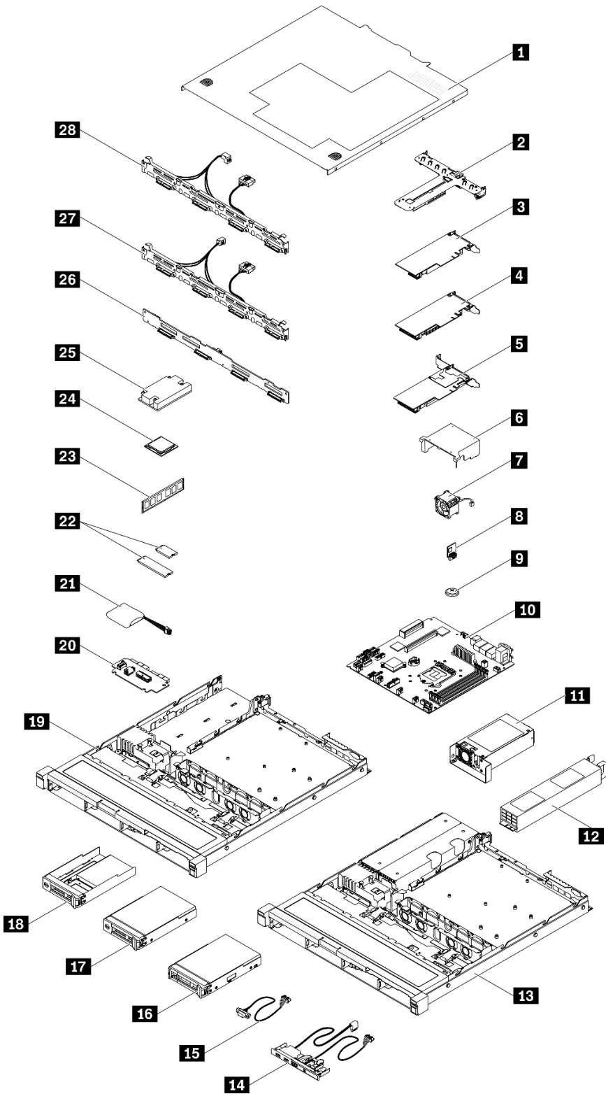
그림 40. 서버 구성 요소 - 3.5인치 드라이브 모델
