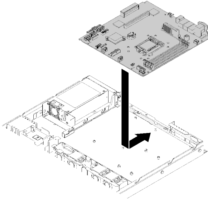
그림 123. 시스템 보드 설치
