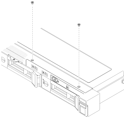
그림 75. 앞면 오퍼레이터 패널 제거
