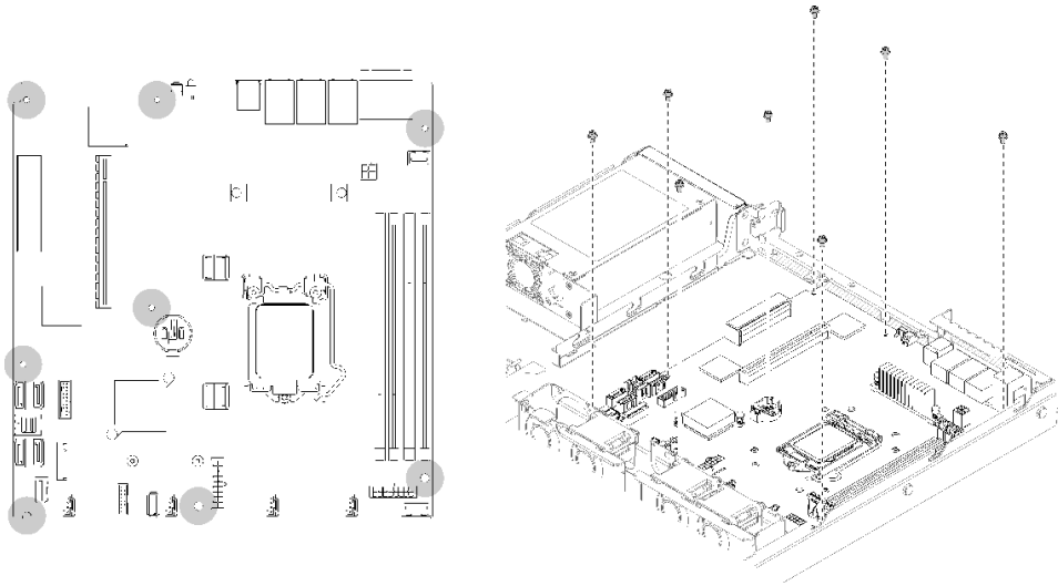
그림 121. 시스템 보드 나사 위치
