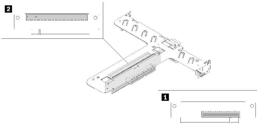
그림 24. x8/x8 나비 라이저 어셈블리
