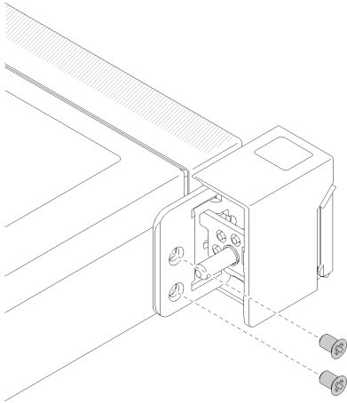
그림 113. 랙 래치 설치
