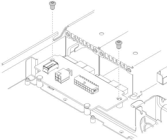
그림 102. 나사 설치
