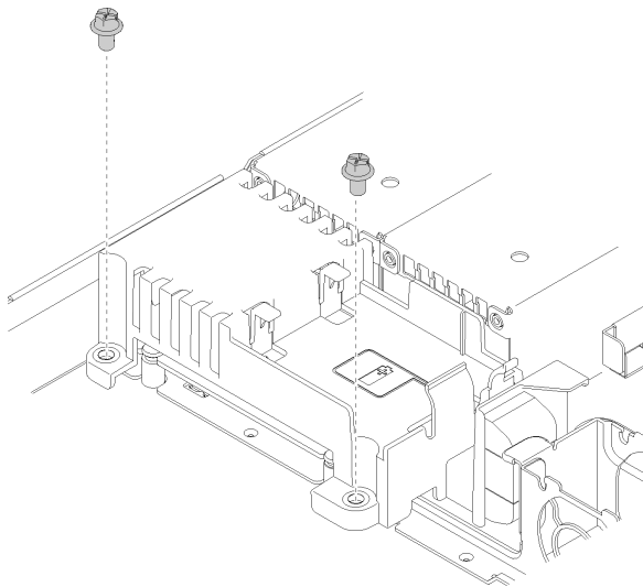
그림 104. 덮개 나사 설치
