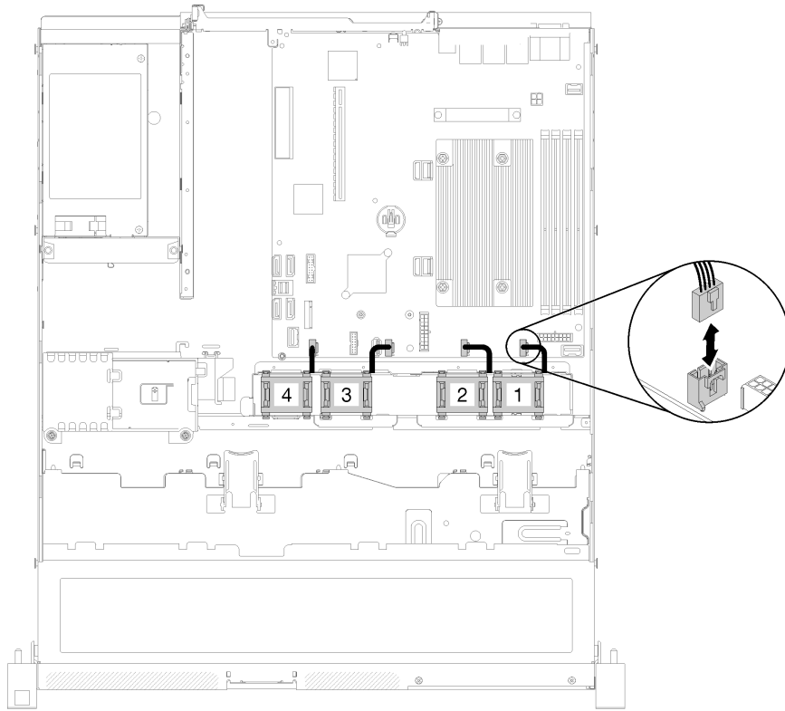
그림 27. 팬 케이블 배선
