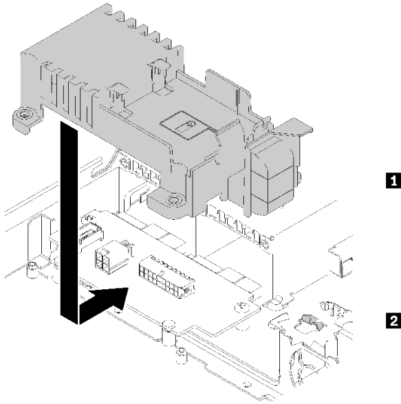
그림 103. 전원 인터페이스 보드 덮개 설치
