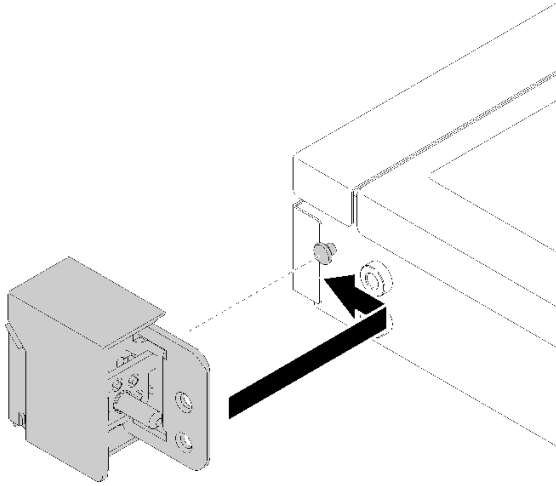
그림 112. 랙 래치 설치
