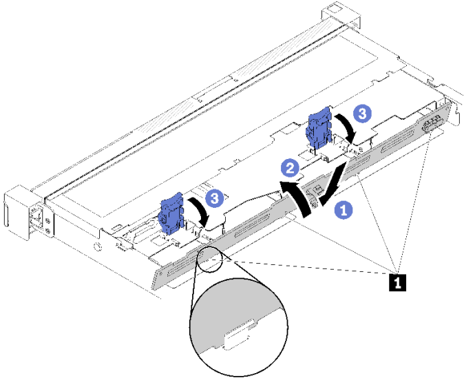
그림 50. 백플레이트 설치
