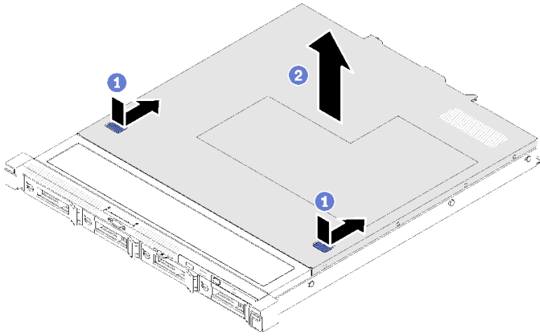
그림 125. 윗면 덮개 제거
