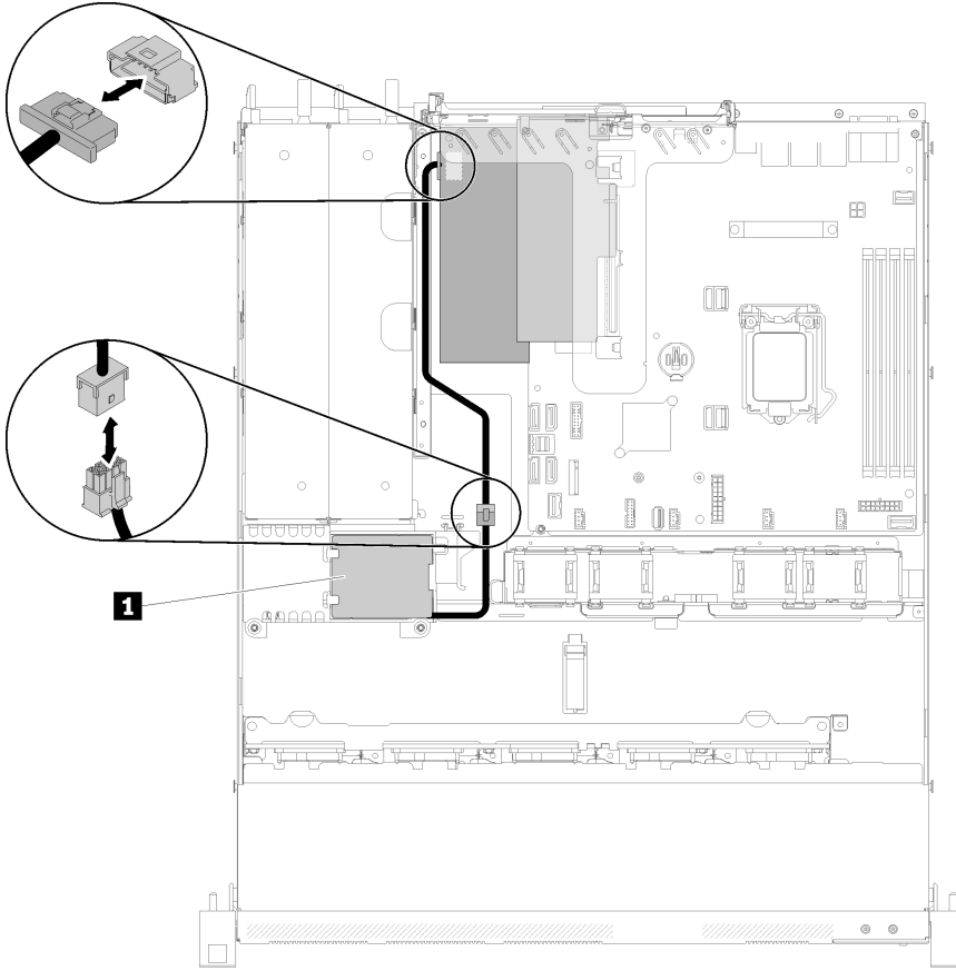
그림 30. 플래시 전원 모듈 케이블 배선
