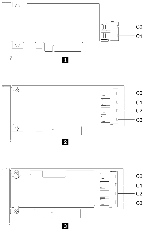
그림 16. RAID 어댑터 및 NVMe 스위치 카드의 커넥터
