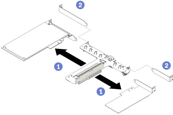
그림 41. 어댑터 제거
