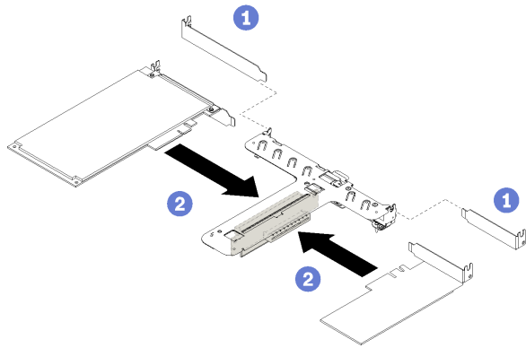
그림 42. 어댑터 설치
