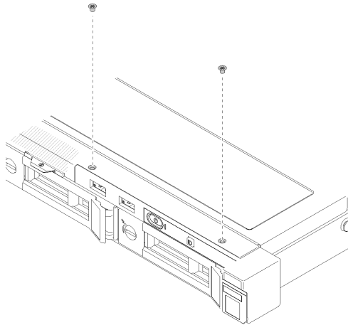
그림 78. 앞면 오퍼레이터 패널(3.5인치 HDD 모델) 설치
