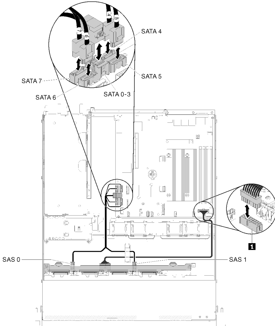
그림 35. 소프트웨어 RAID가 있는 8개의 2.5인치 핫 스왑 드라이브 모델
