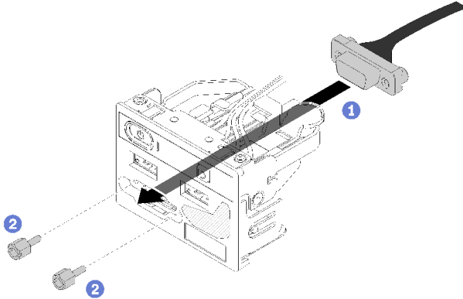
그림 130. VGA 케이블 설치
