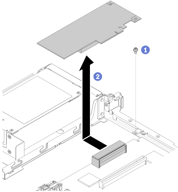
그림 115. RAID 어댑터 제거
