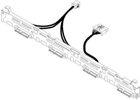
그림 17. 백플레이트, 4개의 3.5인치 심플 스왑 드라이브(RAID x30 어댑터에 연결)
