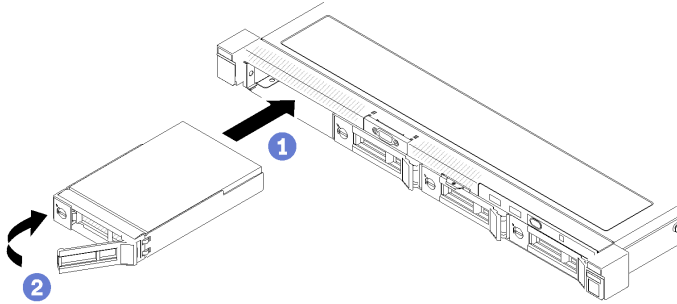
그림 58. 핫 스왑 드라이브 설치
