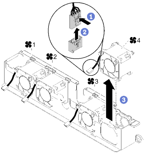
그림 63. 팬 제거
