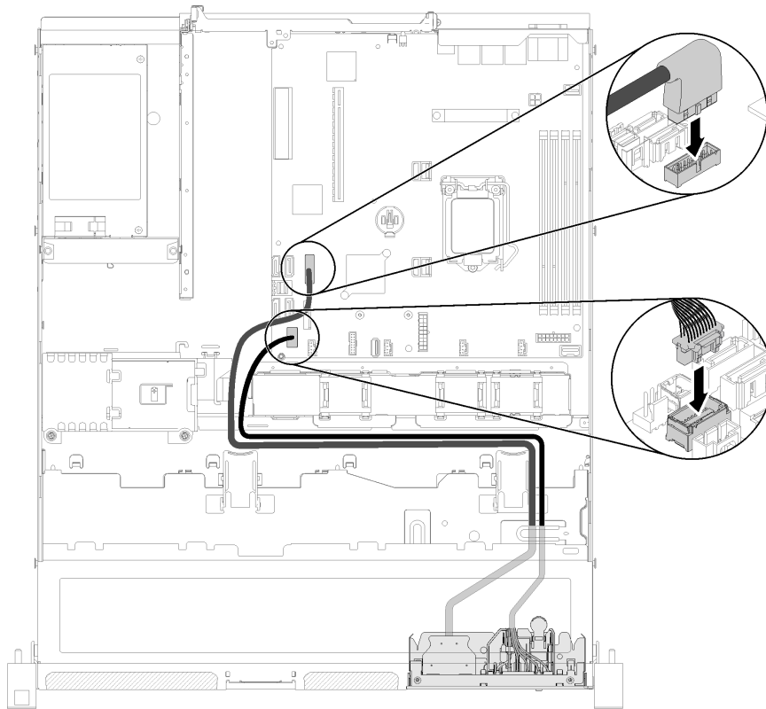
그림 79. 앞면 오퍼레이터 패널 설치
