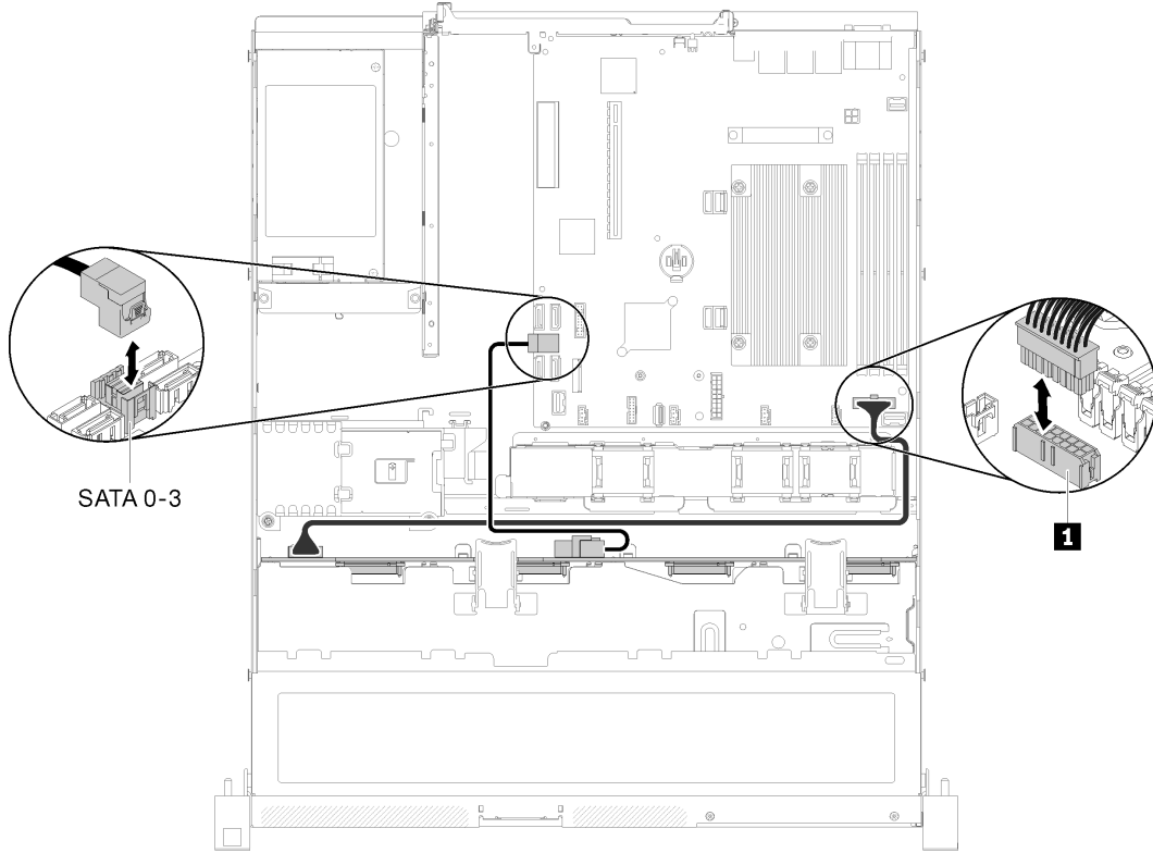
그림 33. 소프트웨어 RAID가 있는 4개의 3.5인치 핫 스왑 드라이브 모델
