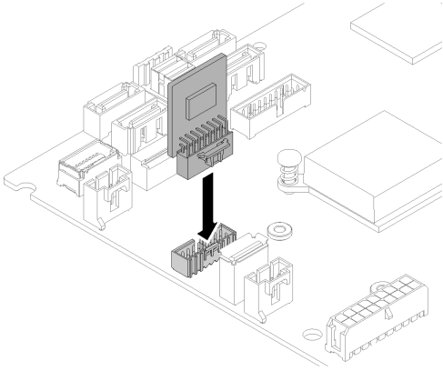
그림 128. TPM 카드(중국 본토만 해당) 설치
