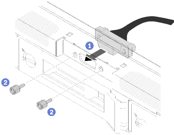
그림 134. VGA 케이블 설치
