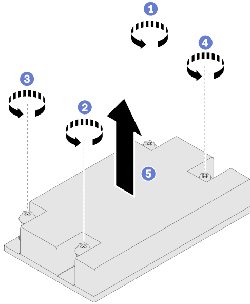
그림 80. 방열판 제거
