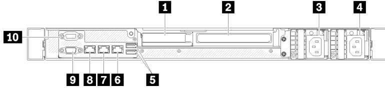
그림 12. 뒷면 보기 - 중복 전원 공급 장치 모델
