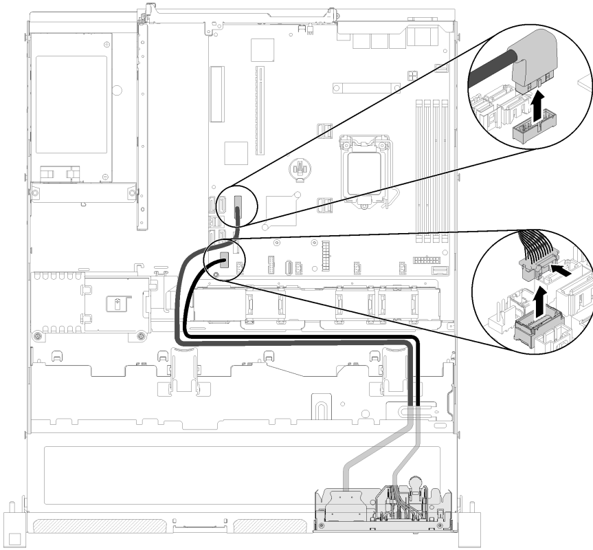
그림 74. 앞면 오퍼레이터 패널(3.5인치 HDD 모델) 제거
