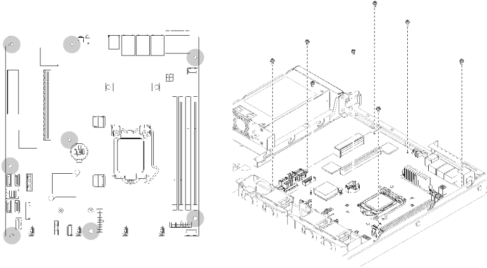
그림 124. 시스템 보드 나사 위치
