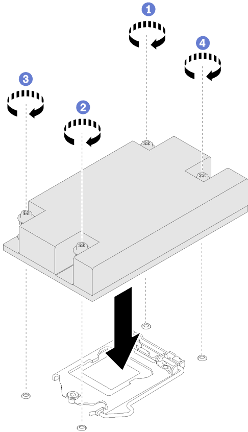
그림 81. 방열판 설치
