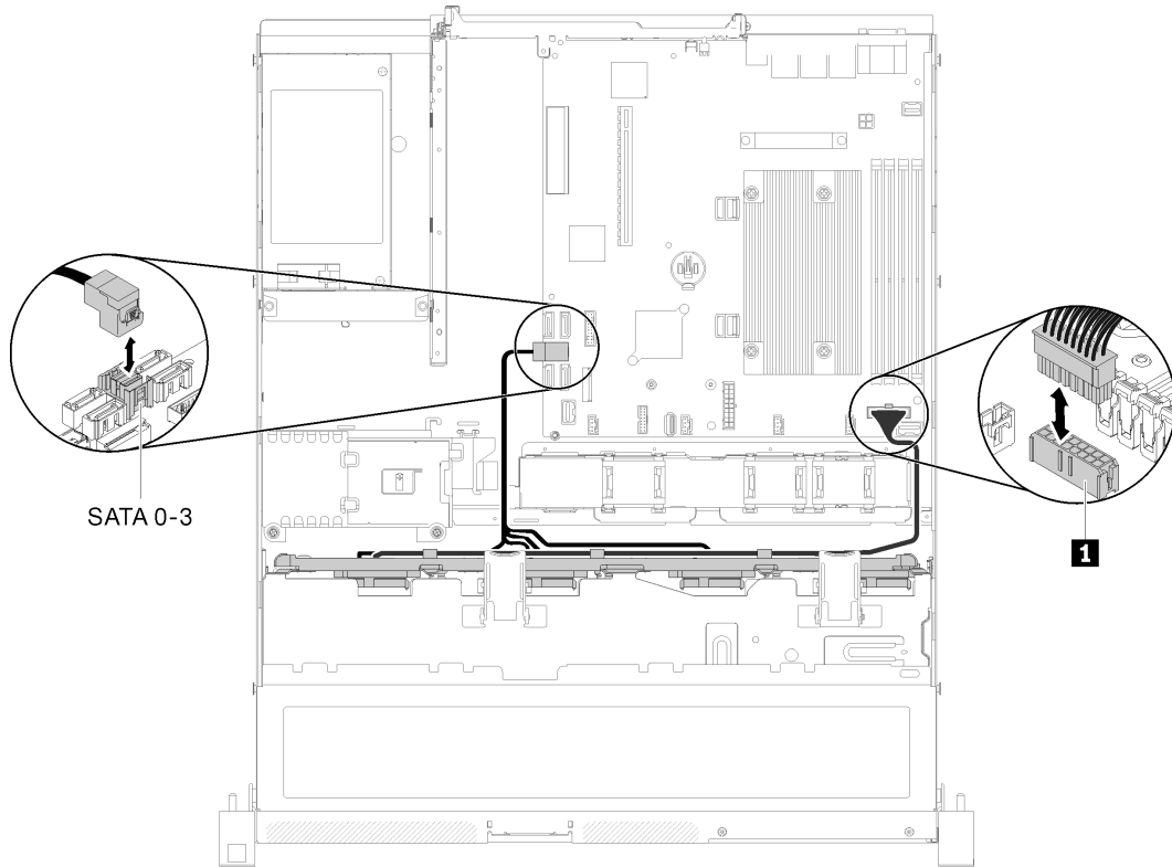
그림 31. 소프트웨어 RAID가 있는 3.5인치 심플 스왑 드라이브 모델
