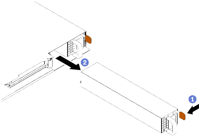
그림 94. 핫 스왑 전원 공급 장치
