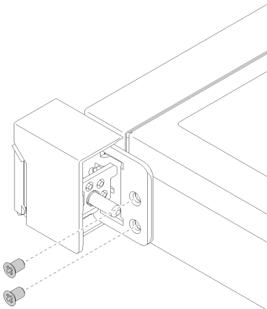
그림 110. 랙 래치 제거
