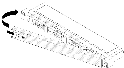
그림 119. 보안 베젤 설치
