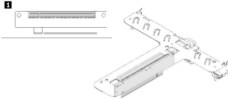
그림 23. x16 PCIe 라이저 어셈블리
