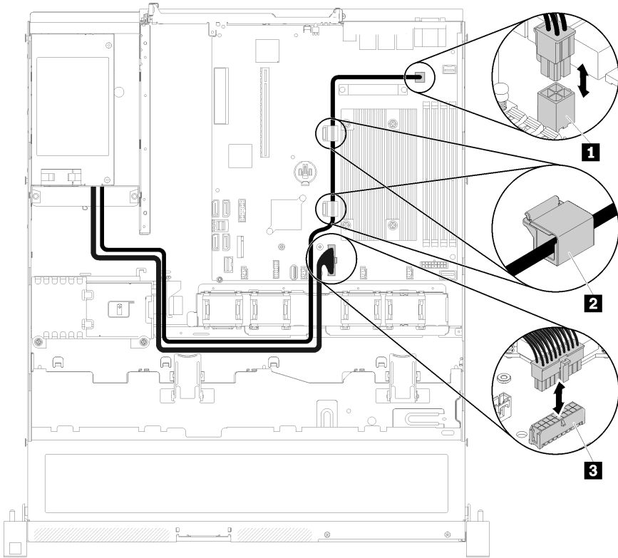
그림 28. 고정 전원 공급 장치 케이블 배선
