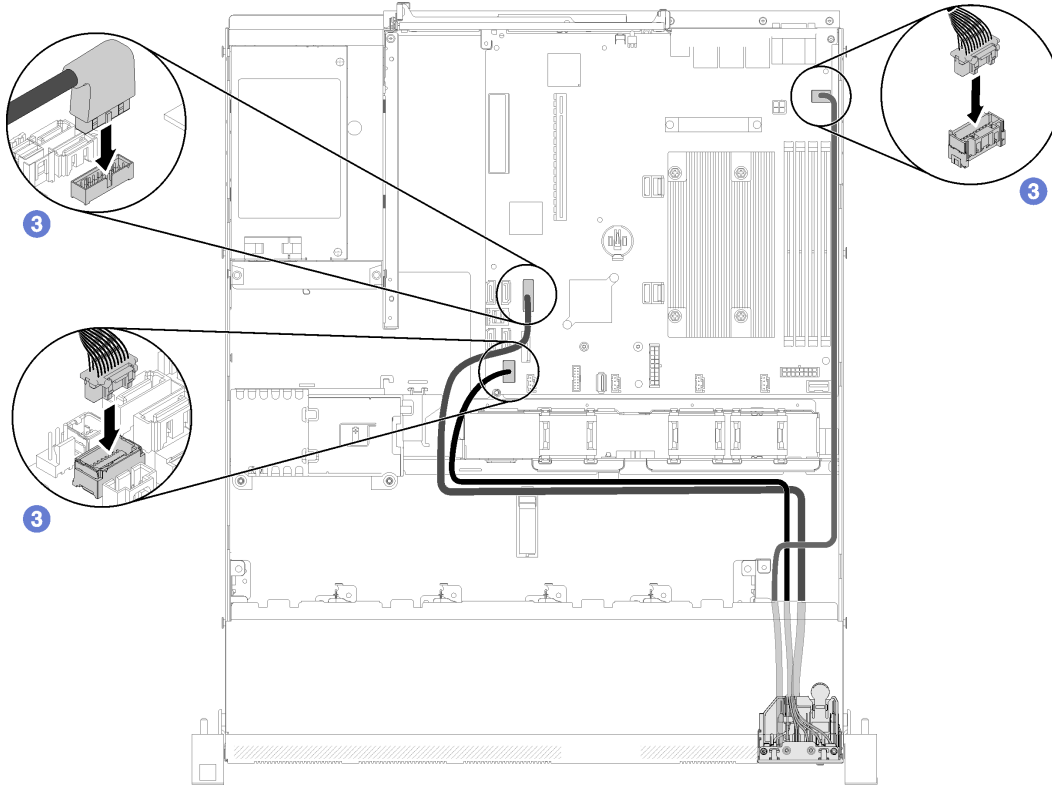
그림 73. 앞면 오퍼레이터 패널(2.5인치 HDD 모델) 케이블 배선
