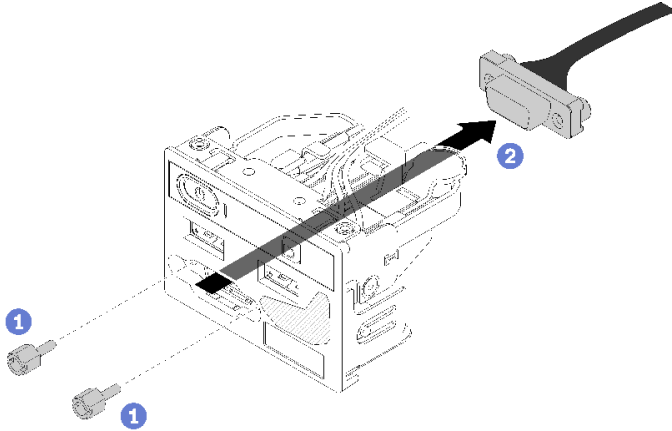
그림 129. VGA 케이블 제거 - 2.5인치 HDD 모델
