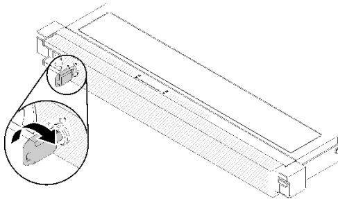
그림 117. 보안 베젤 잠금 해제
