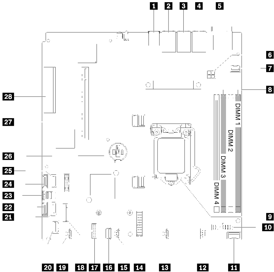
그림 14. 시스템 보드 커넥터
