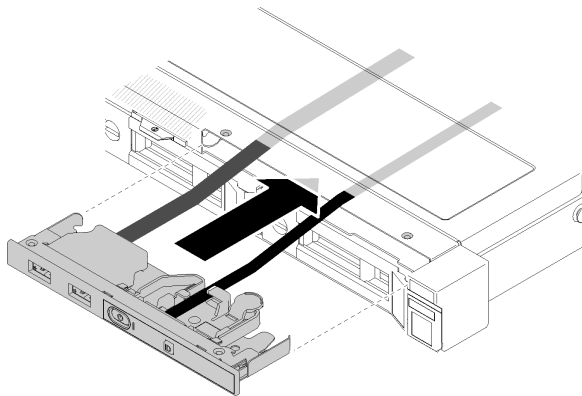
그림 77. 앞면 오퍼레이터 패널(3.5인치 HDD 모델) 설치
