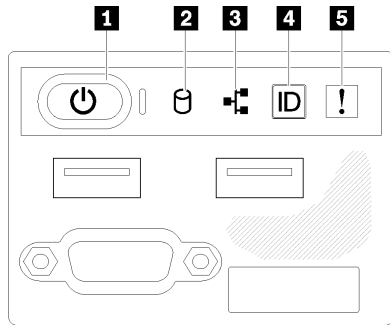
그림 139. 2.5인치 드라이브 새시 앞면 오퍼레이터 패널
