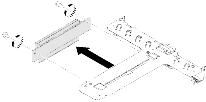
그림 88. PCIe 라이저 카드 제거
