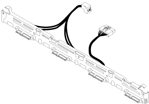
그림 19. 백플레이트, 4개의 3.5인치 심플 스왑 드라이브(온보드 커넥터에 연결)
