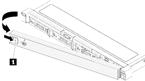
그림 118. 보안 베젤 제거
