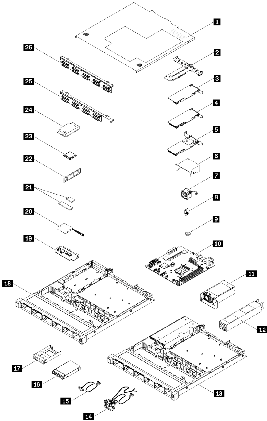
그림 39. 서버 구성 요소 - 2.5인치 드라이브 모델
