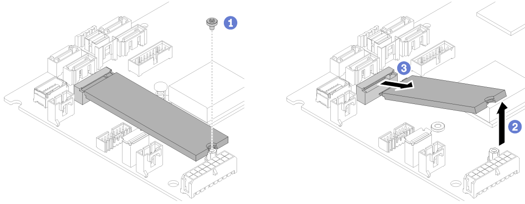
그림 83. M.2 드라이브 제거
