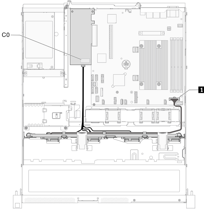
그림 32. 하드웨어 RAID가 있는 3.5인치 심플 스왑 드라이브 모델
