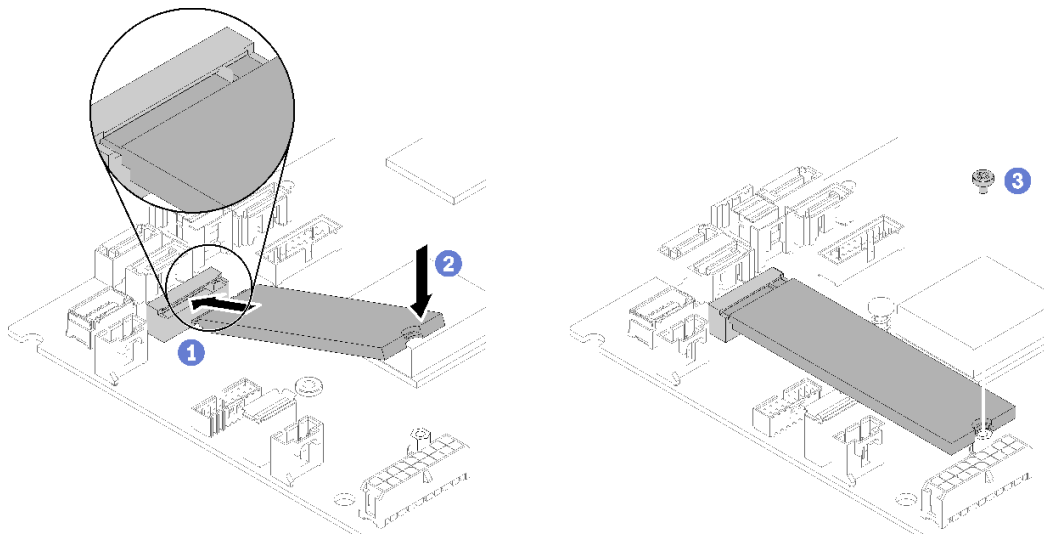
그림 86. M.2 드라이브 설치
