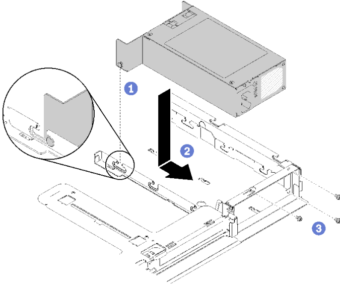
그림 93. 전원 공급 장치 설치
