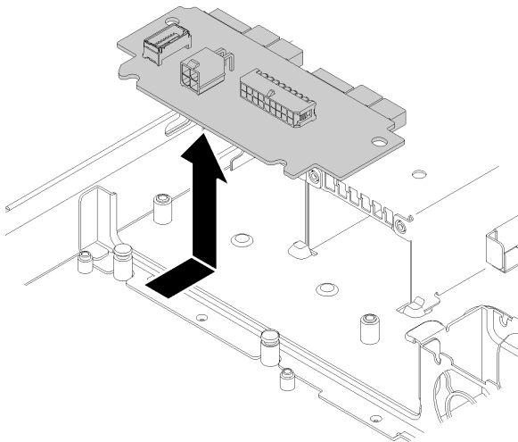
그림 100. 전원 인터페이스 보드 제거
