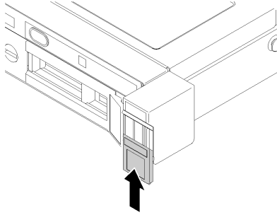
그림 114. ID 레이블 설치
