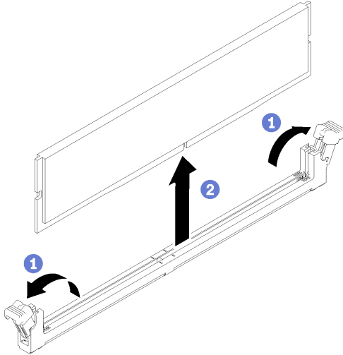
그림 54. DIMM 제거
