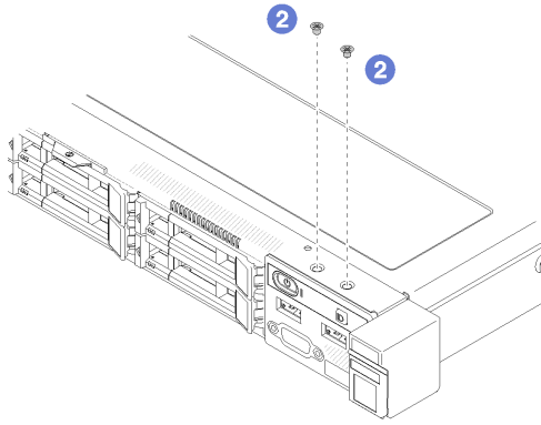
그림 69. 나사 제거
