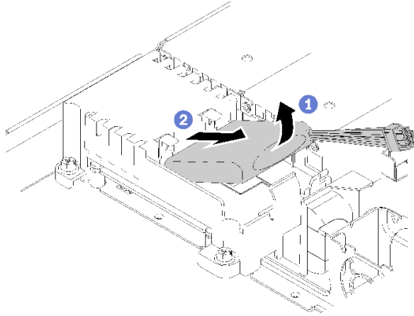
그림 66. 플래시 전원 모듈 제거
