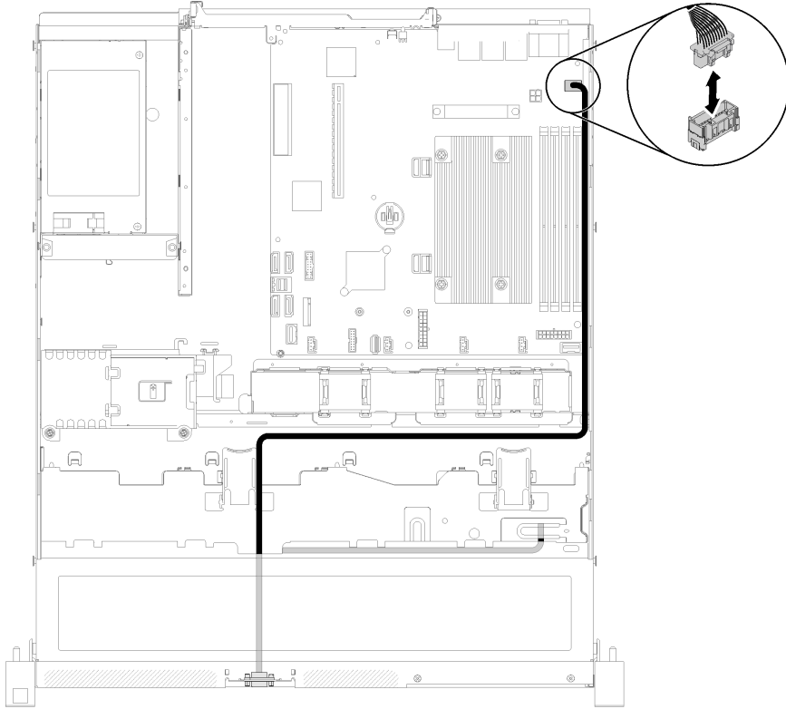
그림 25. 4개의 드라이브가 있는 앞면 VGA 케이블 배선
