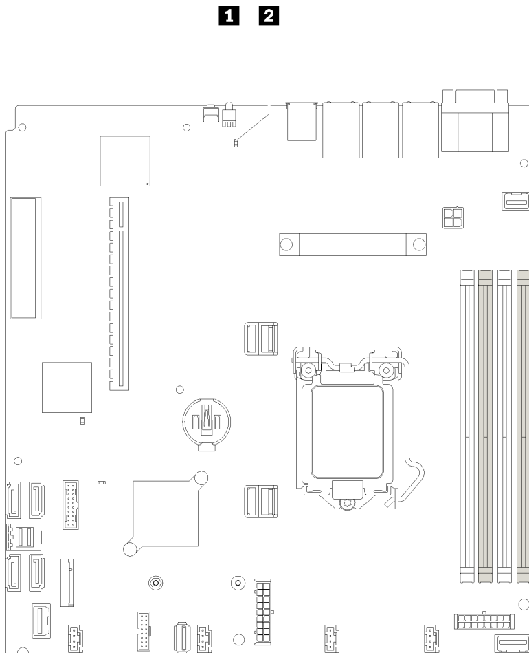
그림 143. 시스템 보드 LED
