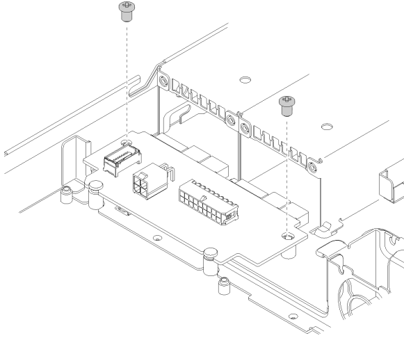
그림 99. 전원 인터페이스 보드 나사 제거
