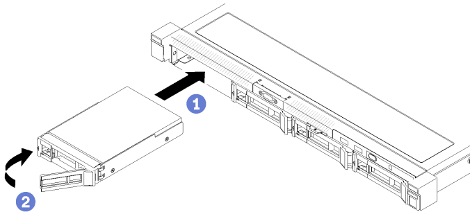
그림 62. 3.5인치 핫 스왑 드라이브 설치
