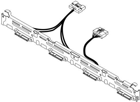
그림 18. 백플레이트, 4개의 3.5인치 심플 스왑 드라이브(RAID x40 어댑터에 연결)
