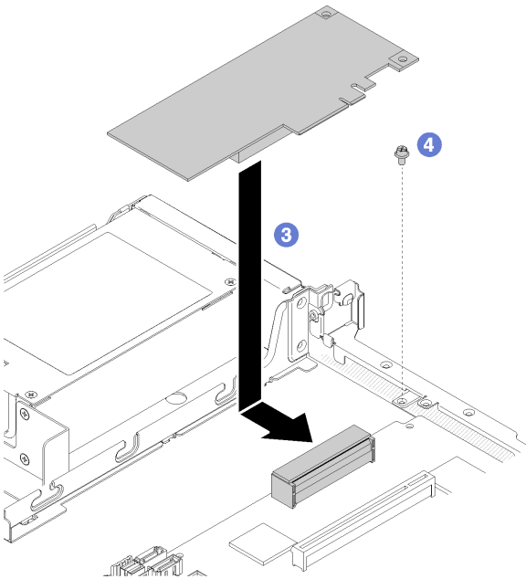
그림 116. RAID 어댑터 설치
