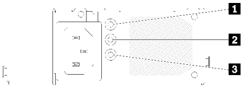
그림 141. 300W 전원 공급 장치 LED
