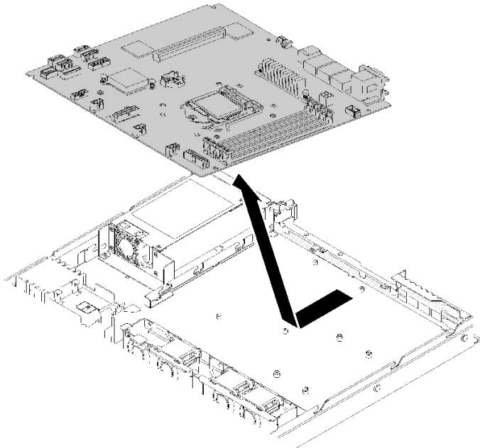
그림 122. 시스템 보드 제거
