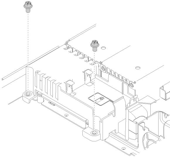
그림 97. 덮개 나사 제거
