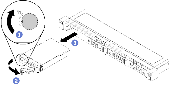
그림 57. 심플 스왑 드라이브 제거
