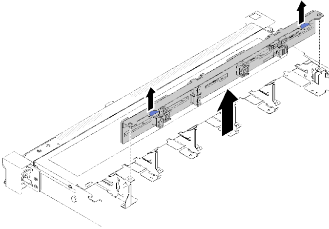
그림 45. 2.5인치 핫 스왑 드라이브 백플레인 제거
