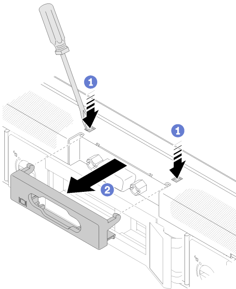
그림 132. VGA 케이블 제거
