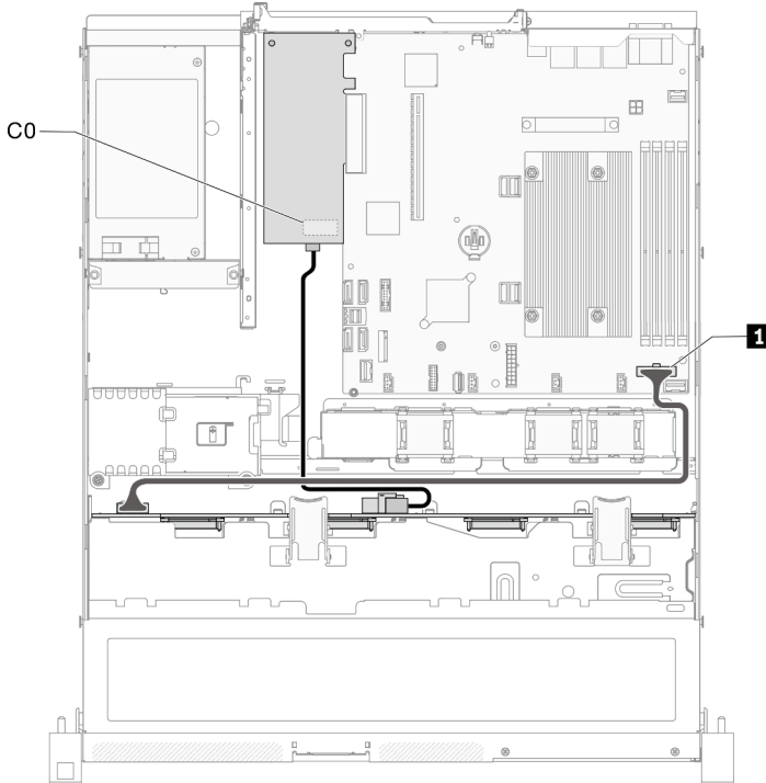
그림 34. 하드웨어 RAID가 있는 4개의 3.5인치 핫 스왑 드라이브 모델
