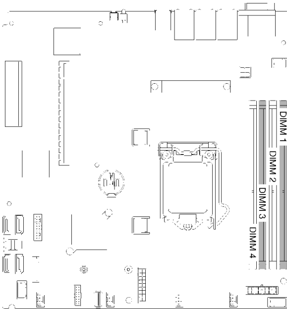
그림 53. DIMM 커넥터
