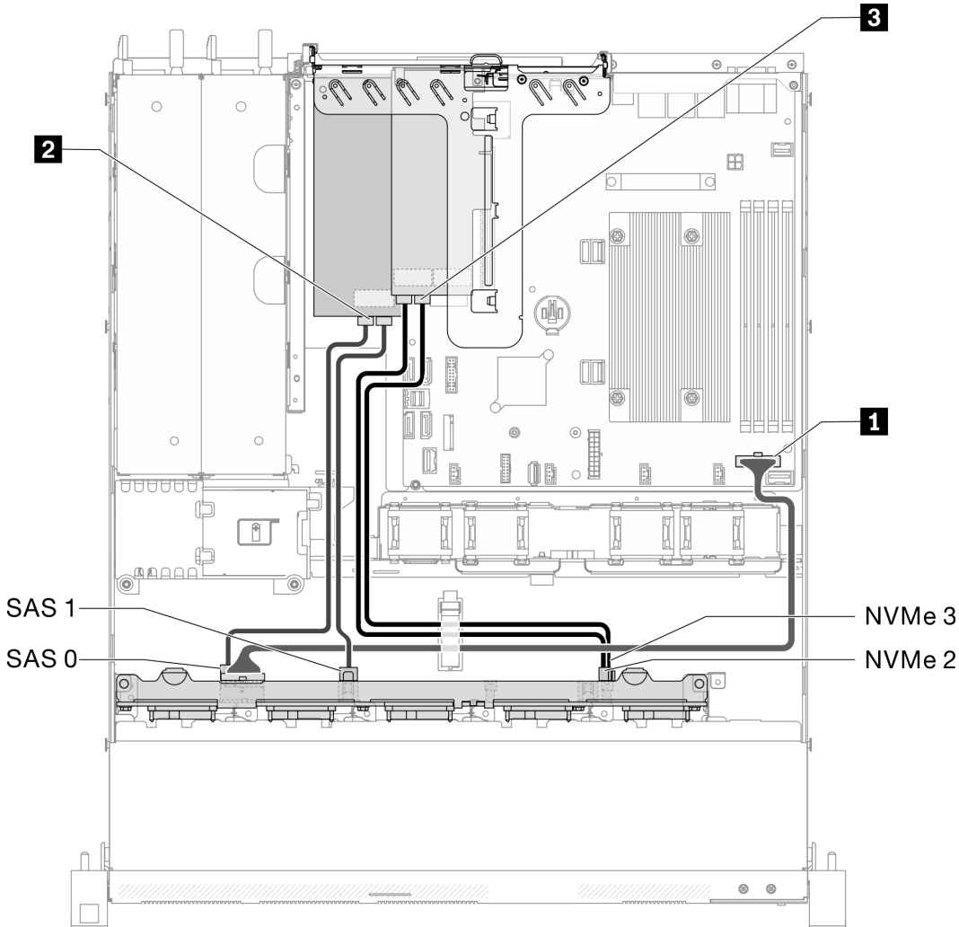
그림 38. 10개의 2.5인치 핫 스왑 드라이브 모델(2개의 NVMe 드라이브 지원)
