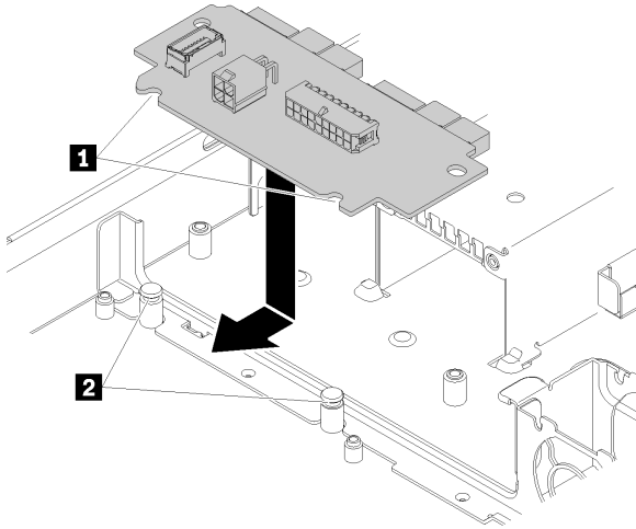
그림 101. 전원 인터페이스 보드 설치
