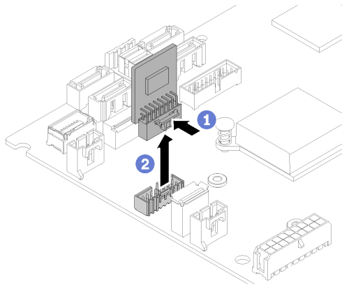
그림 127. TPM 카드(중국 본토만 해당) 제거
