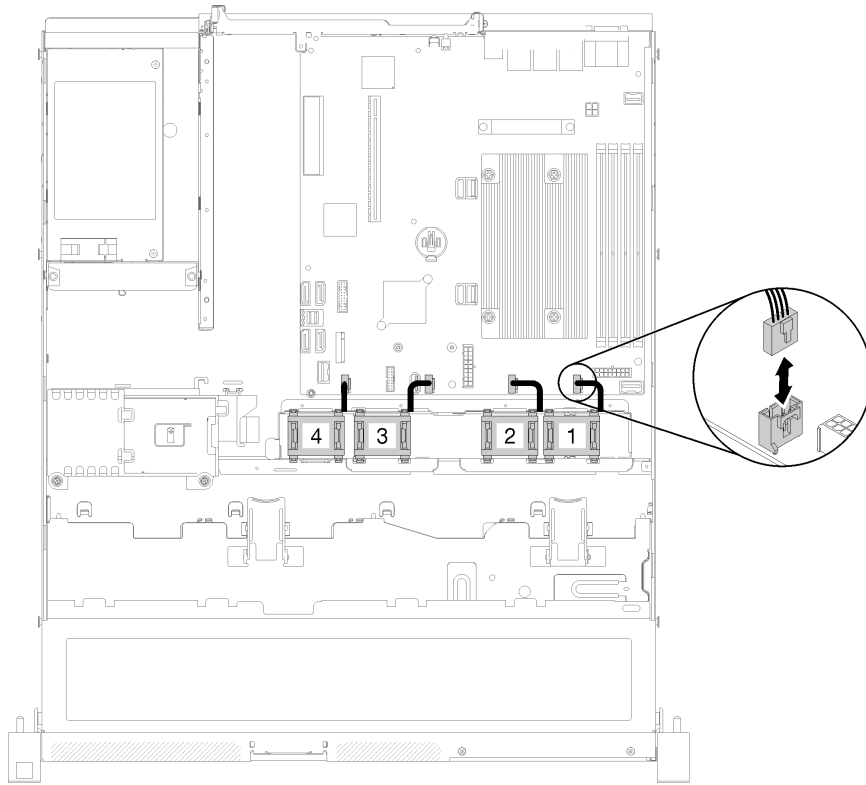
그림 65. 팬 전원 케이블 배선
