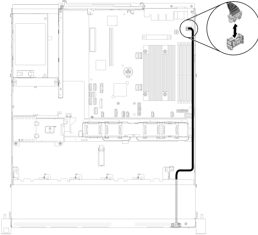
그림 26. 10개의 드라이브가 있는 전면 VGA 케이블 배선
