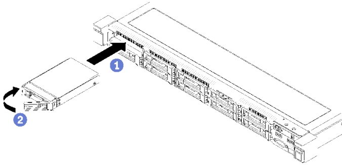
그림 61. 2.5인치 핫 스왑 드라이브 설치
