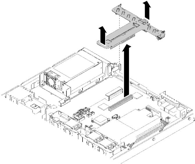
그림 87. PCIe 라이저 어셈블리 제거
