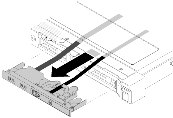
그림 76. 앞면 오퍼레이터 패널 제거
