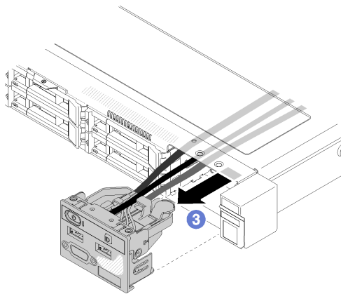
그림 70. 앞면 오퍼레이터 패널 제거
