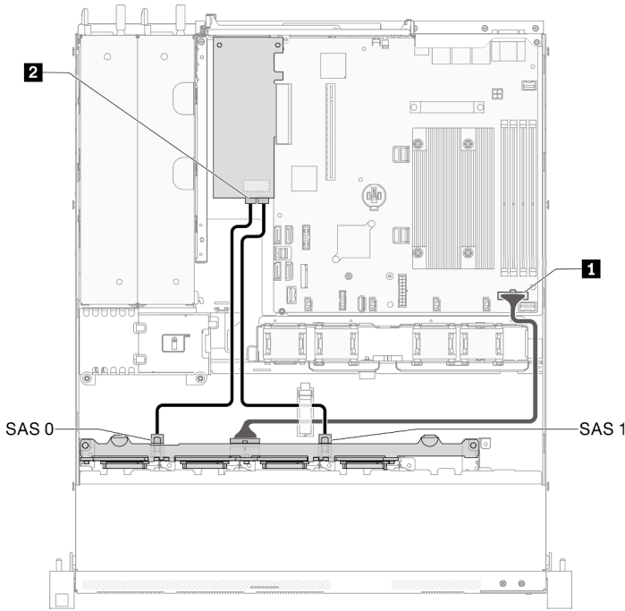
그림 36. 하드웨어 RAID가 있는 8개의 2.5인치 핫 스왑 드라이브 모델
