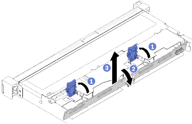
그림 49. 백플레이트 제거
