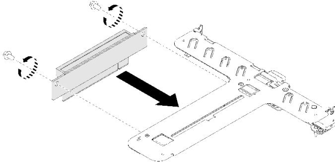
그림 89. PCIe 라이저 카드 설치
