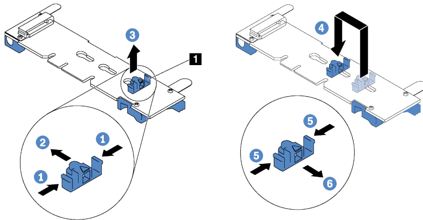
Figura 34. Ajuste del elemento de sujeción M.2
