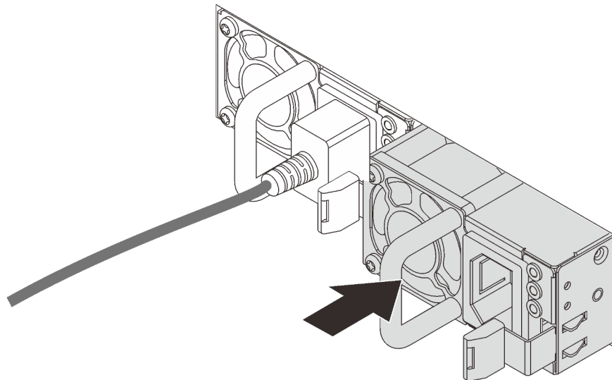
Figura 40. Instalación de una fuente de alimentación de intercambio en caliente
