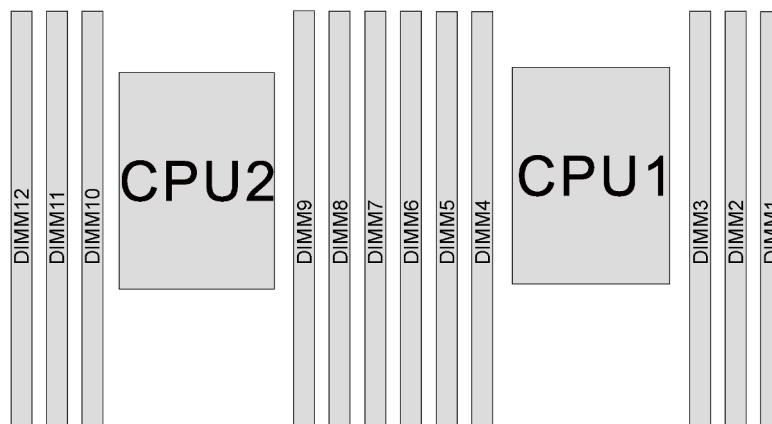
Figura 25. Ranuras de módulos de memoria en la placa del sistema
