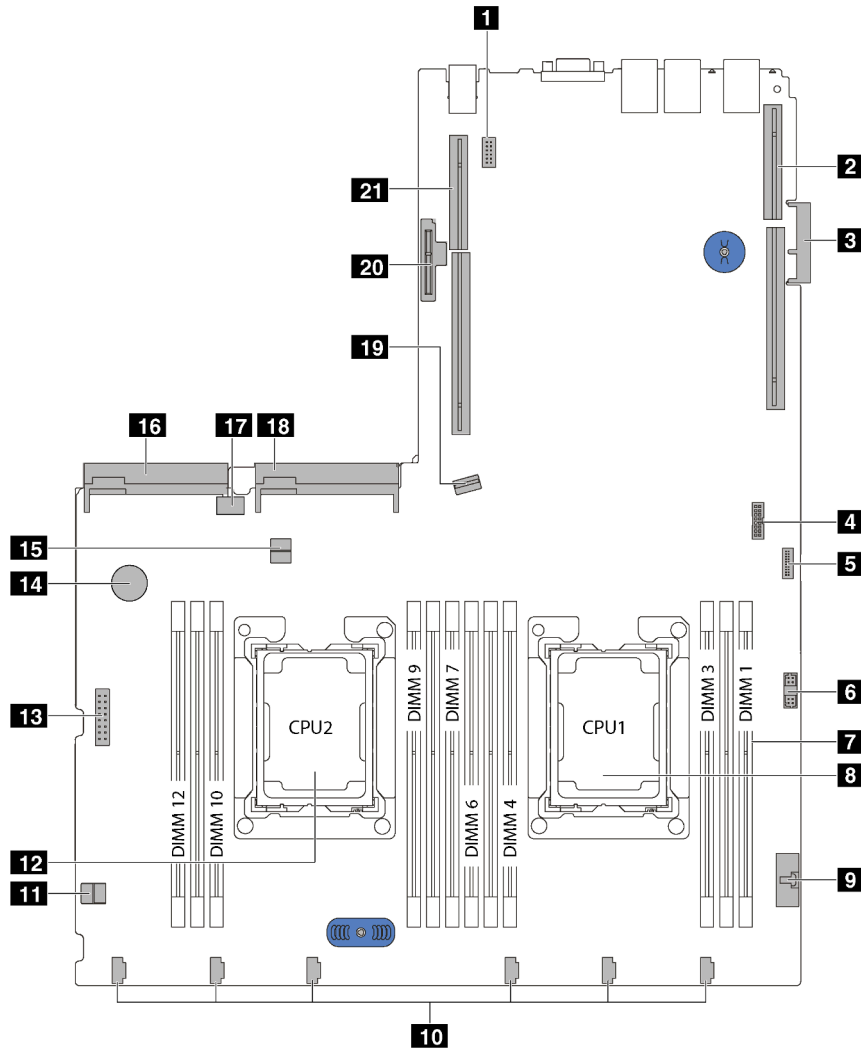
Figura 10. Componentes de la placa del sistema
