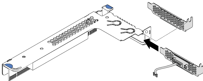
Figura 35. Instalación de módulo de puerto serie
