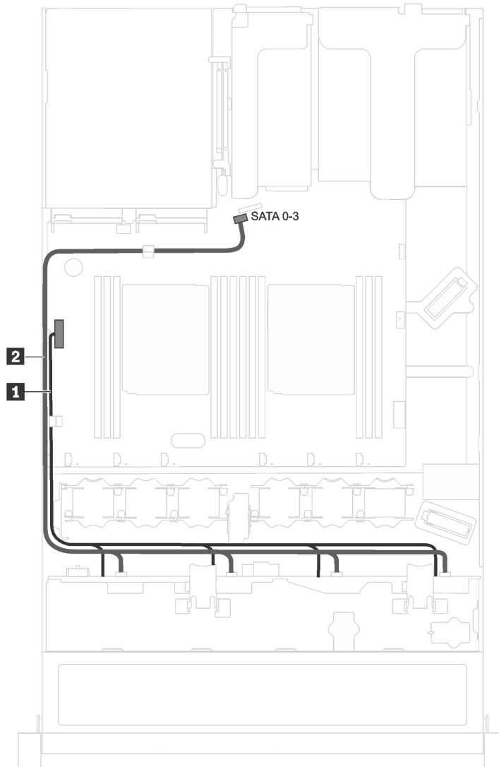
Figura 17. Disposición de cables del modelo de servidor de cuatro unidades de 3,5 pulgadas de intercambio simple
