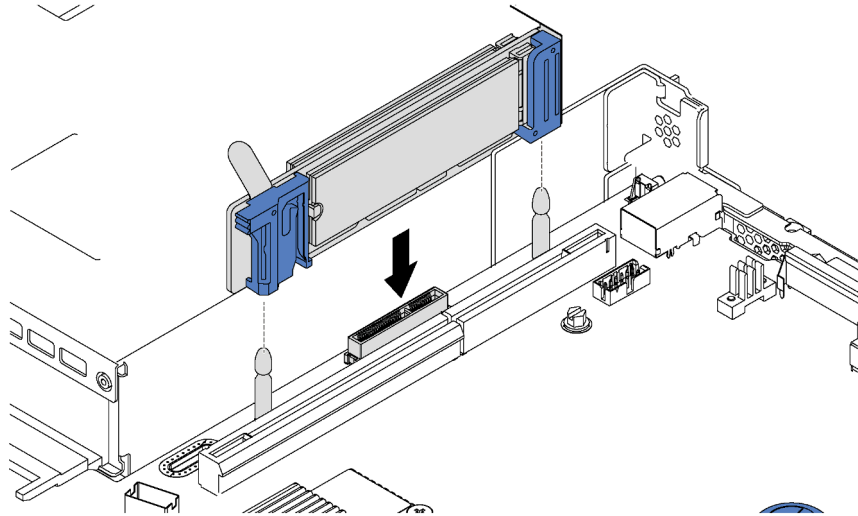
Figure 33. Installation du fond de panier M.2
