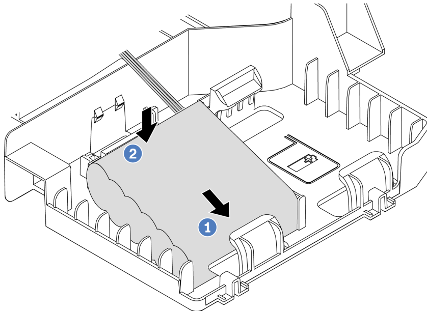
Figure 41. Installation du module de supercondensateur RAID
