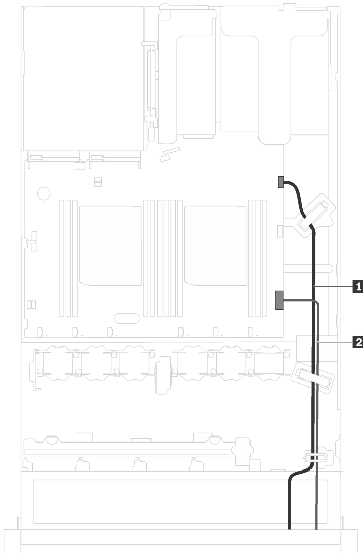
Figure 13. Cheminement des câbles pour le bloc d'E-S avant
