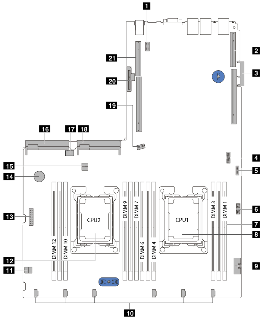
Figure 10. Composants de la carte mère
