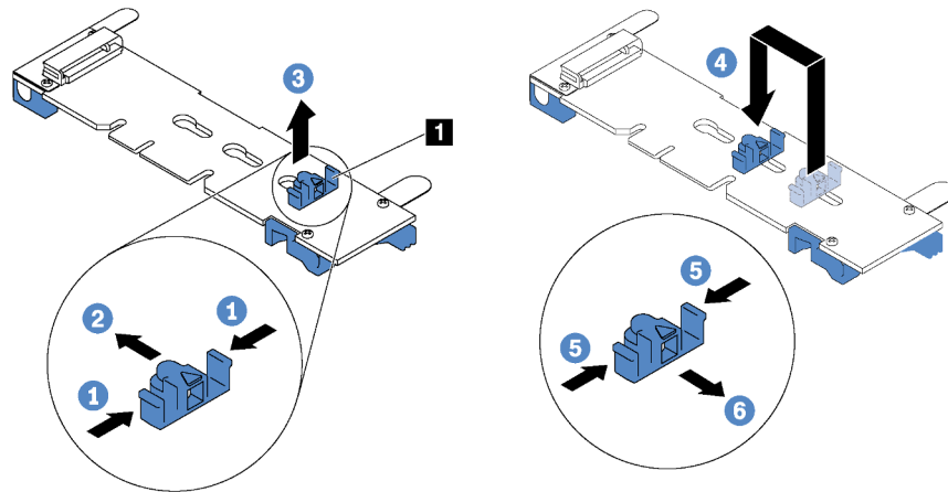
Figure 34. Ajustement du dispositif de retenue M.2
