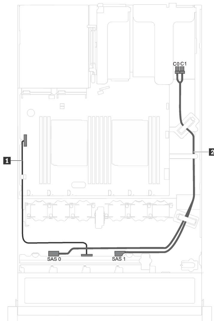
Figure 15. Cheminement des câbles pour le modèle de serveur doté de huit unités remplaçables à chaud 2,5 pouces
