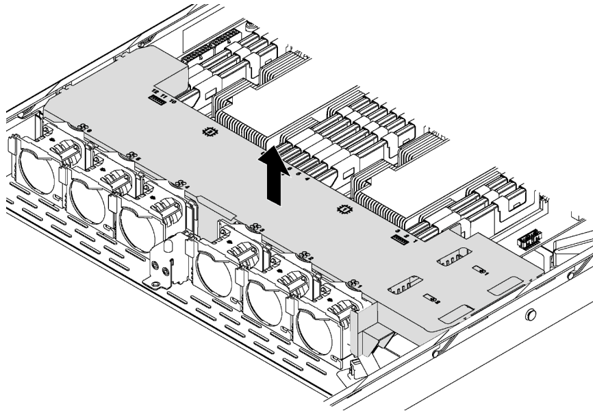
Figure 22. Retrait de la grille d'aération
