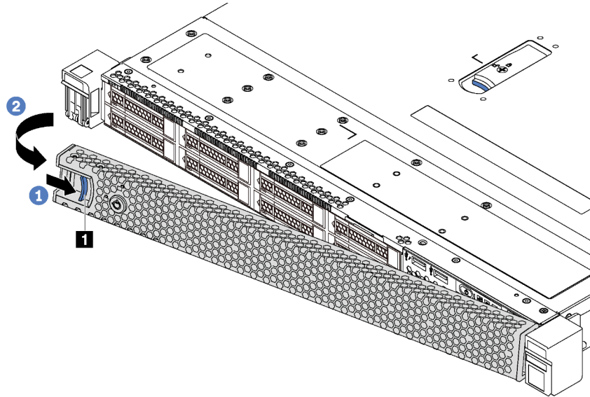
Figure 20. Retrait du panneau de sécurité
