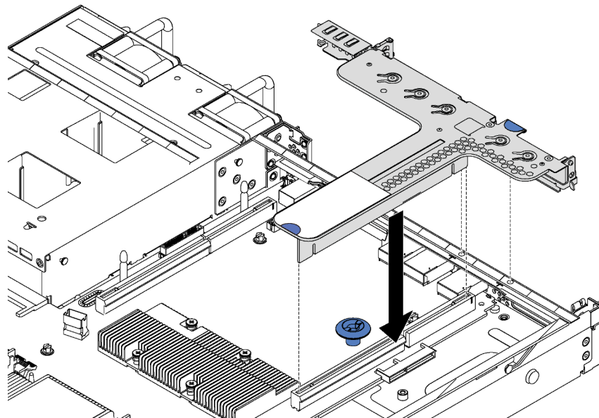
Figure 30. Installation de l'assemblage de cartes mezzanines
