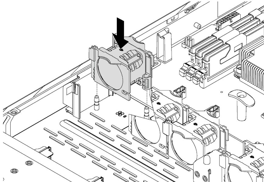
Figure 26. Installation du ventilateur système
