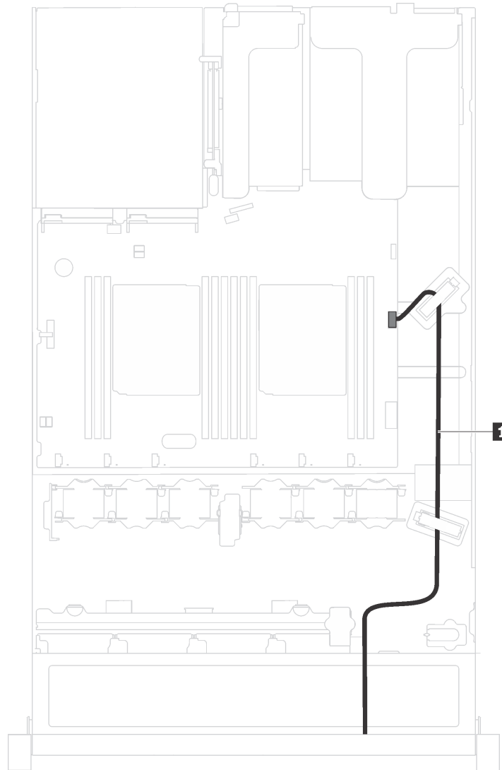
Figure 12. Cheminement des câbles du connecteur VGA
