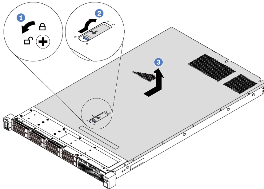
Figure 21. Retrait du carter supérieur
