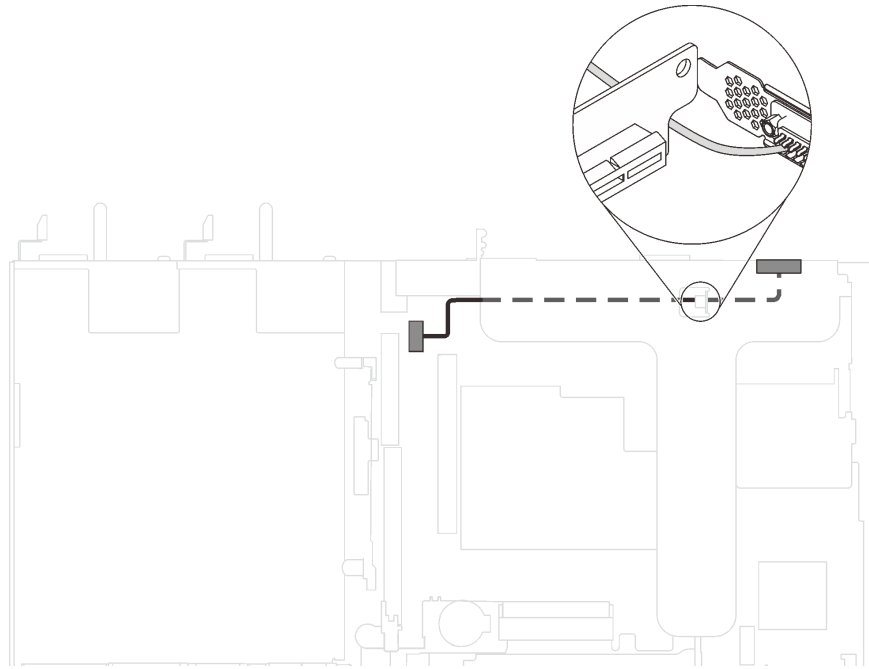
Figure 36. Cheminement des câbles pour le module de port série installé dans l'emplacement PCIe 1
