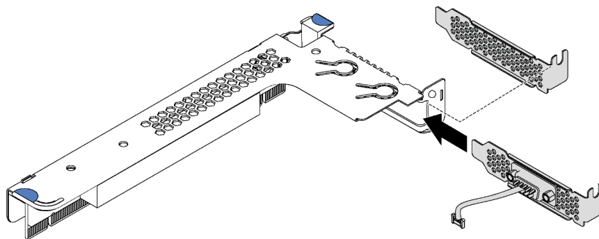
Figure 35. Installation du module de port série
