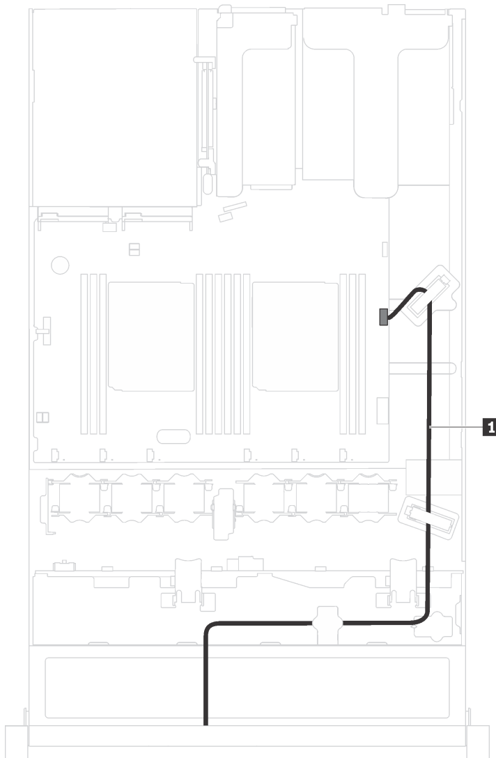
Figure 11. Cheminement des câbles du connecteur VGA
