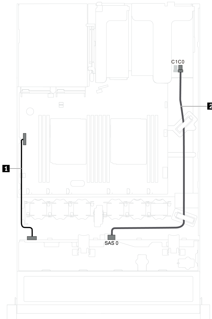
Figure 16. Cheminement des câbles pour le modèle de serveur doté de quatre unités remplaçables à chaud 3,5 pouces
