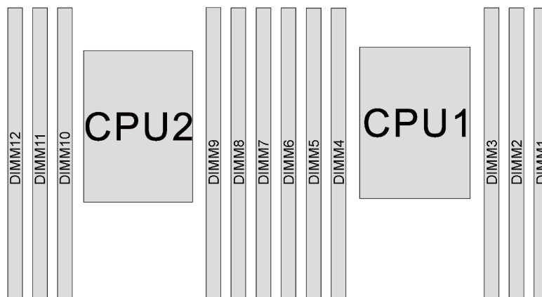
Figure 25. Emplacements de module de mémoire sur la carte mère
