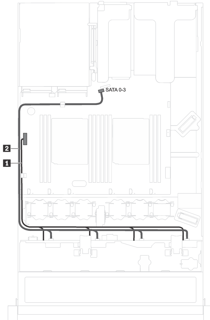
Figure 17. Cheminement des câbles pour le modèle de serveur doté de quatre unités à remplacement standard 3,5 pouces
