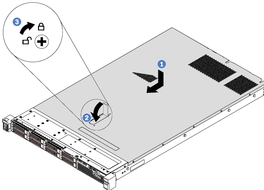
Figure 43. Installation du carter supérieur
