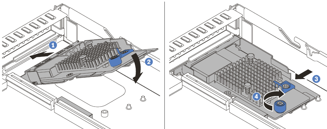
Figure 37. Installation d'adaptateur LOM
