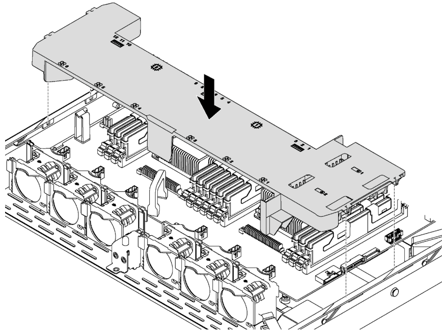
Figure 42. Installation de la grille d'aération
