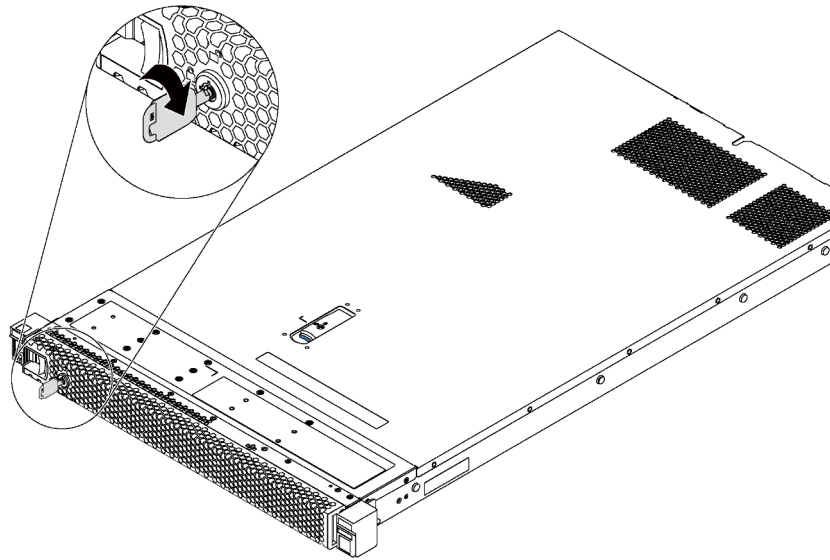
Figure 19. Déverrouillage du panneau de sécurité
