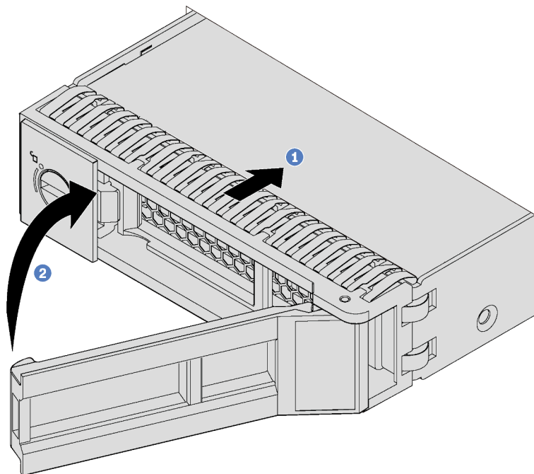
Figure 45. Installation d'une unité à remplacement standard
