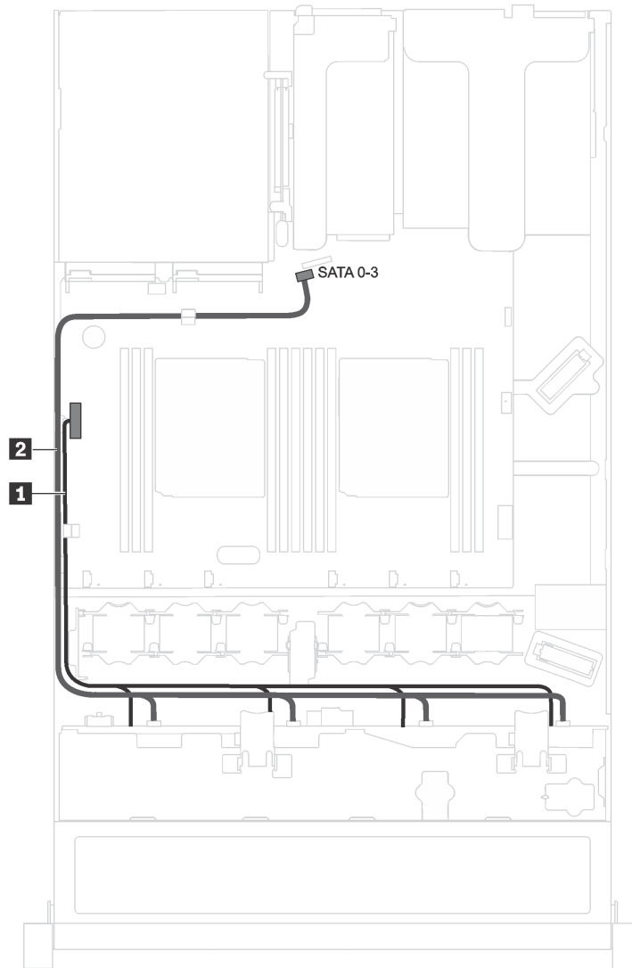
図 19. 4 台の 3.5 型シンプル・スワップ・ドライブを搭載したサーバー・モデルのケーブル配線
