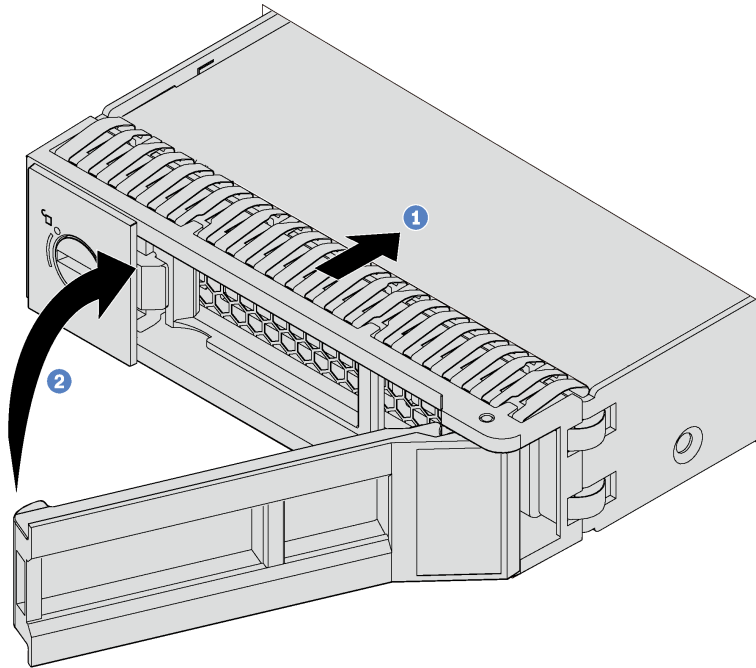
図 55. シンプル・スワップ・ドライブの取り付け
