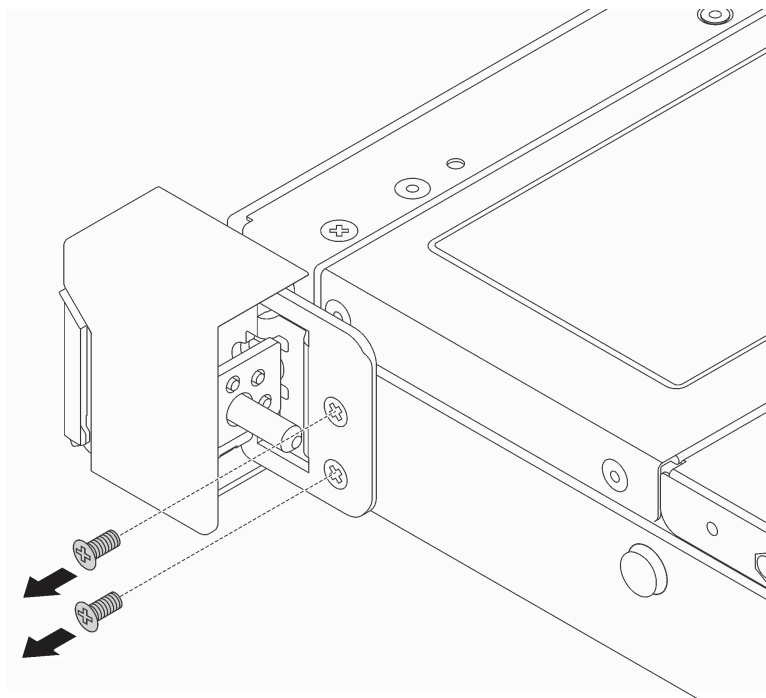
図22. ラック・ラッチのねじの取り外し
