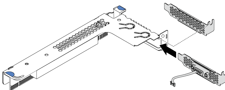
図 88. シリアル・ポート・モジュールの取り付け
