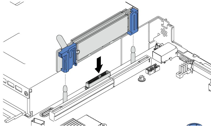
図 85. M.2 バックプレーンの取り付け
