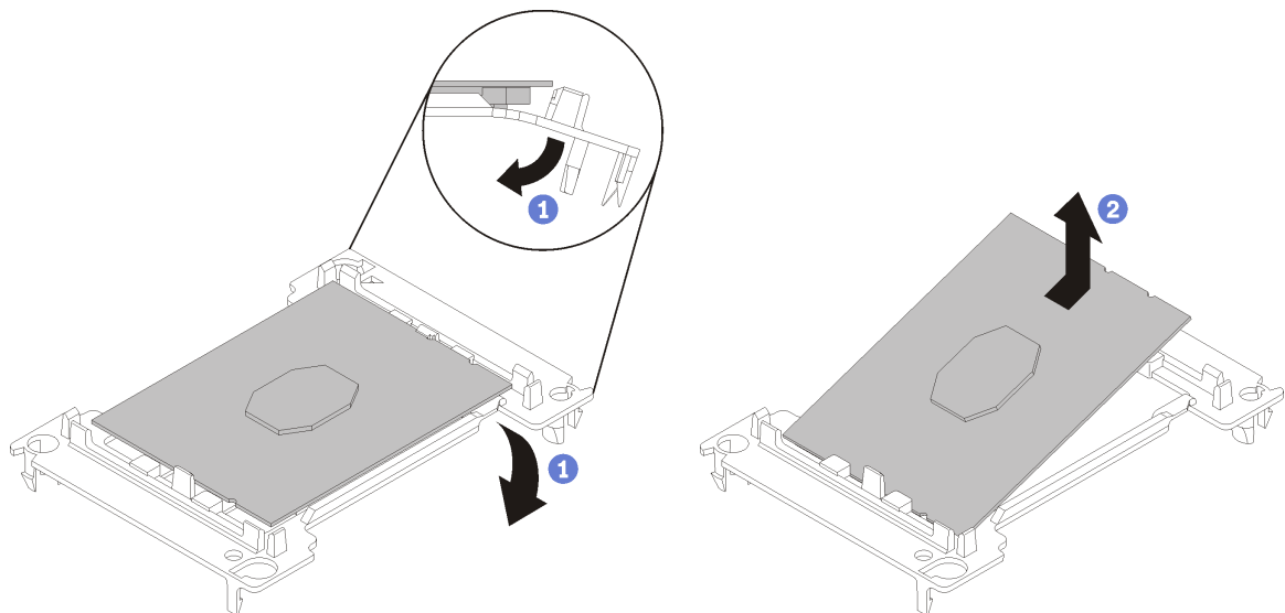
図 94. プロセッサ保持器具の取り外し
