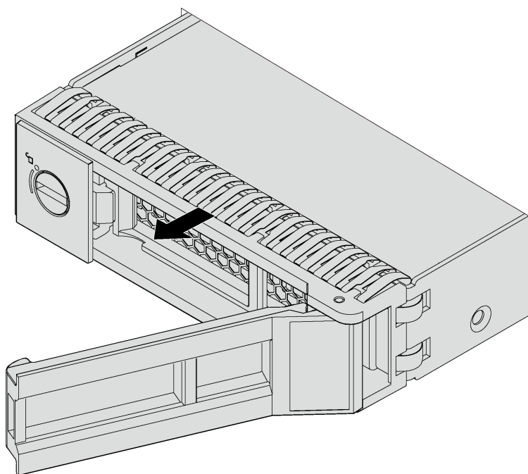
図54. ドライブをドライブ・ベイから引き出す
