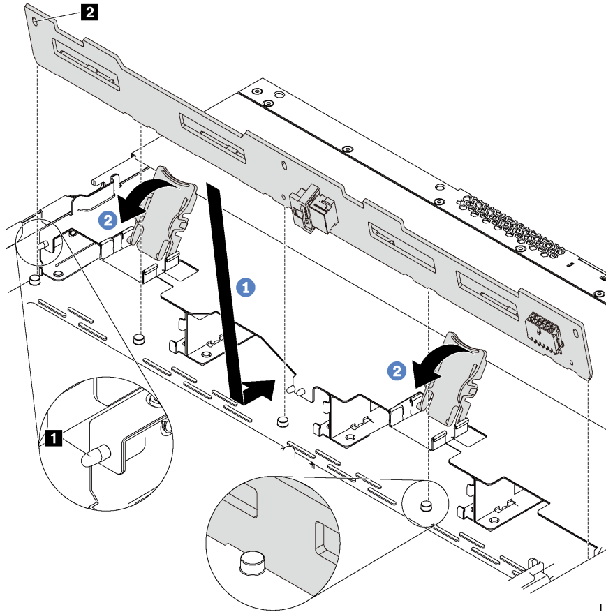
図 45. バックプレーンの取り付け
