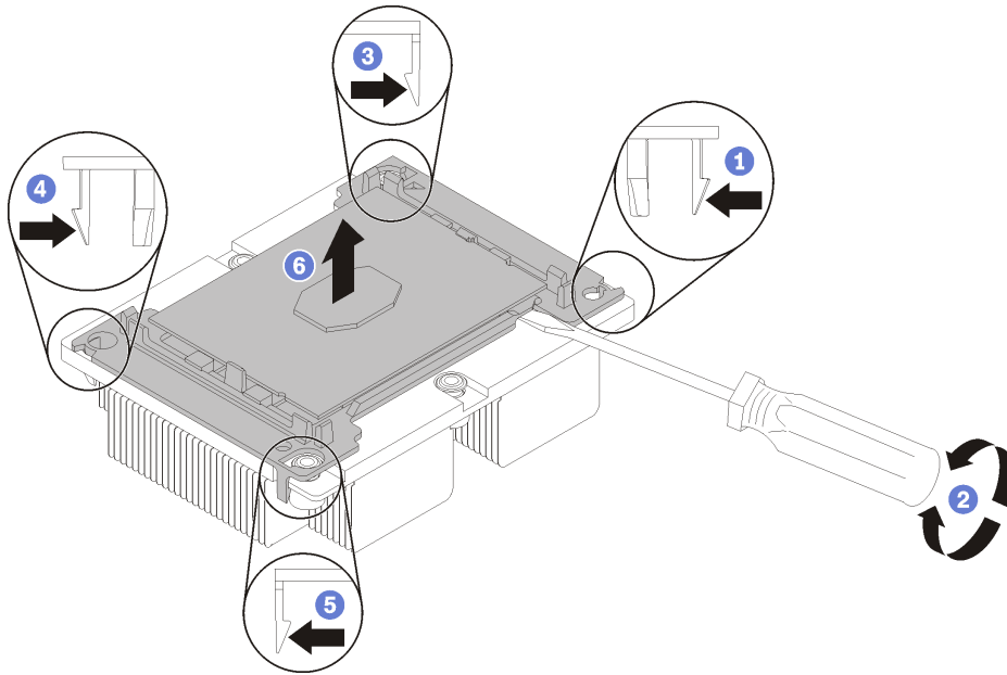
図93. ヒートシンクのプロセッサからの分離
