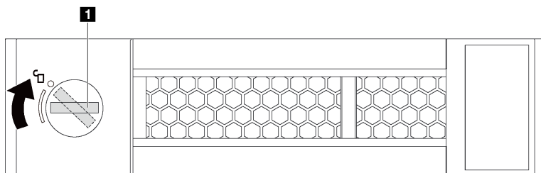
図53. ドライブ・トレイ・ハンドルを開く
