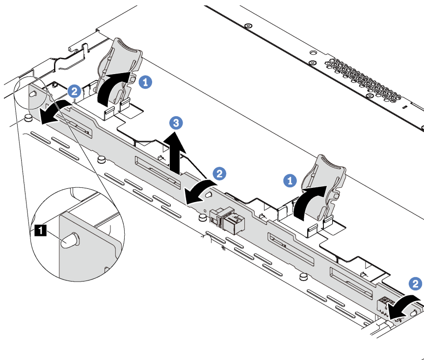
図 44. バックプレーンの取り外し
