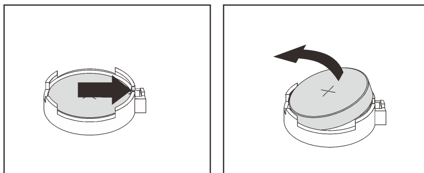
図 59. CMOS バッテリーの取り外し
