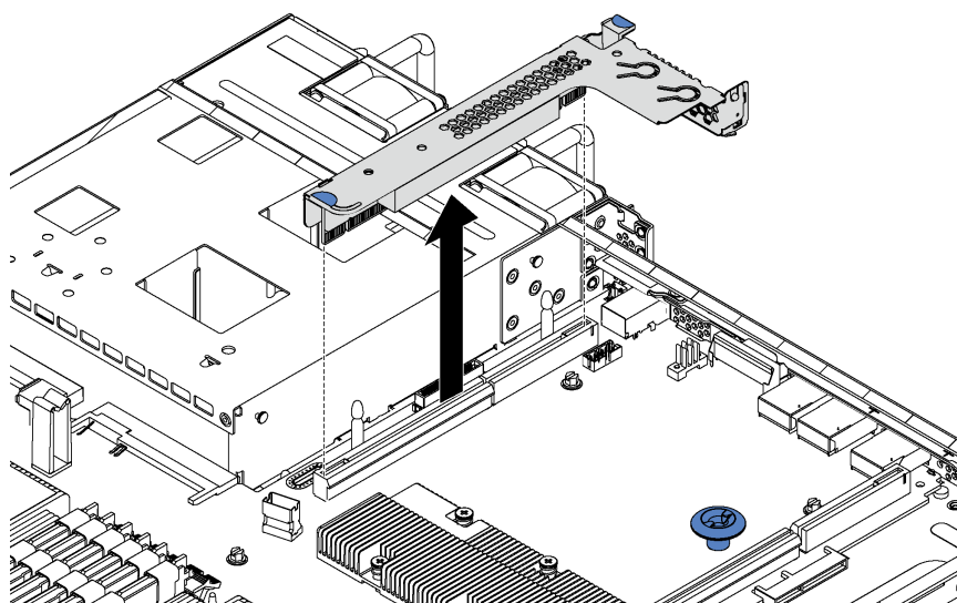
図 86. ライザー・アセンブリーの取り外し
