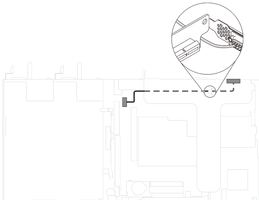
図 89. PCIe スロット 1 に搭載されたシリアル・ポート・モジュールのケーブル配線
