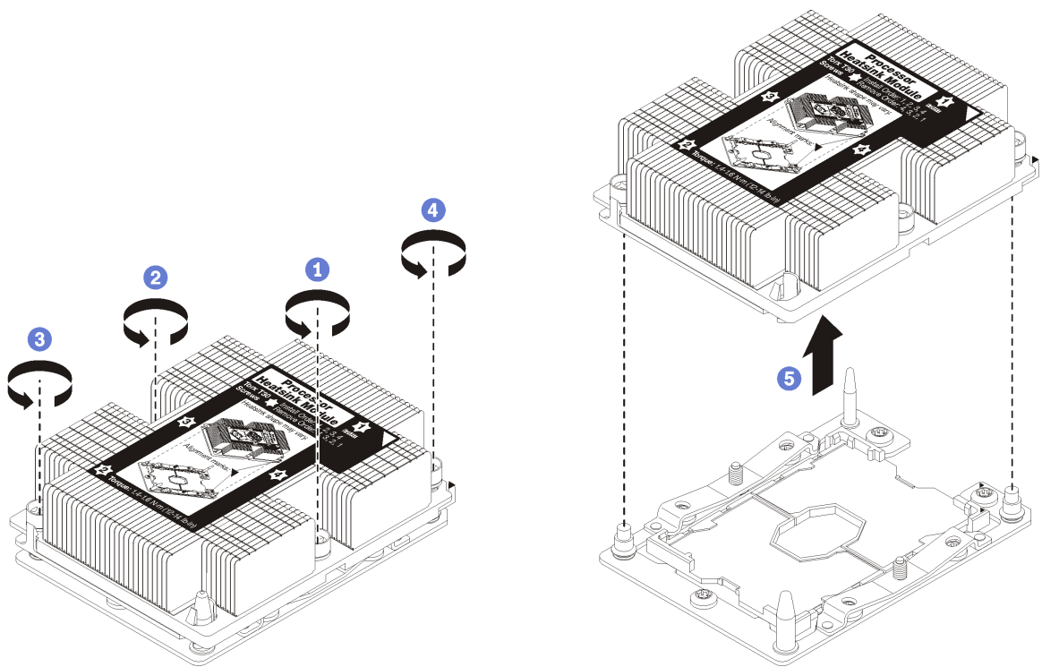
図92. PHM の取り外し
