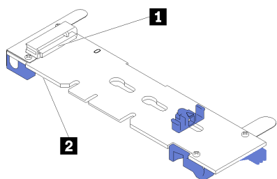
図 83. M.2 ドライブ・スロット
