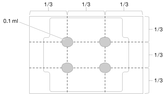
図96. 熱伝導グリースの適切な形
