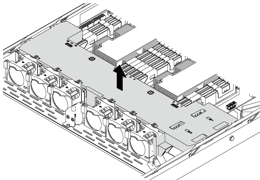
図 34. エアー・バッフルの取り外し
