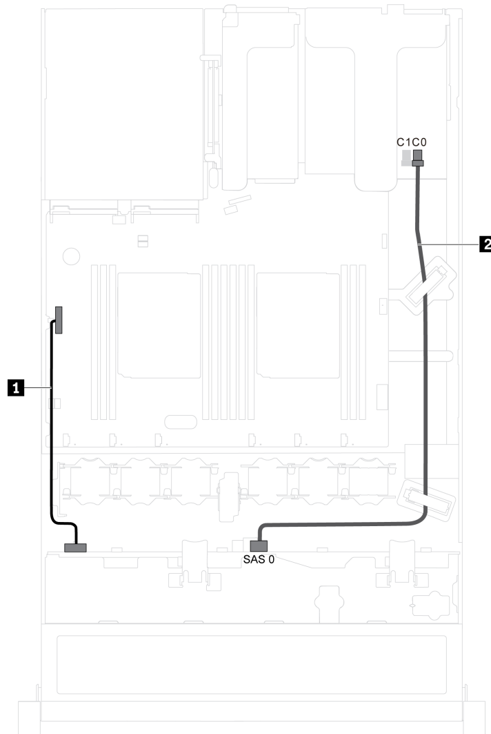
図 18. 4 台の 3.5 型ホット・スワップ・ドライブを搭載したサーバー・モデルのケーブル配線
