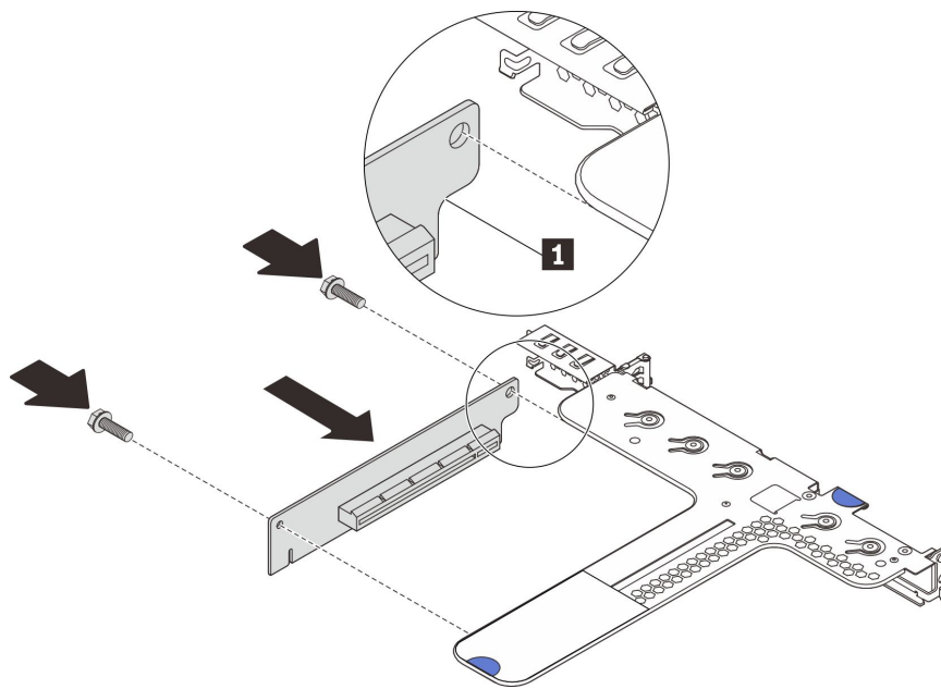
図 78. ライザー・カードの取り付け
