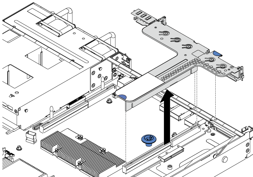
図76. ライザー・アセンブリーの取り外し
