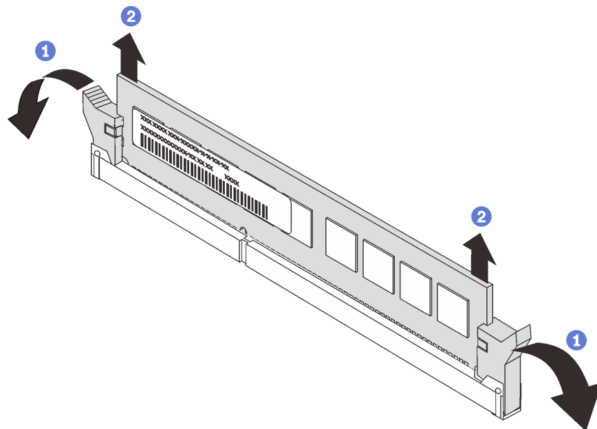
図 56. メモリー・モジュールの取り外し
