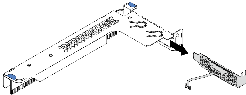
図87. シリアル・ポート・モジュールの取り外し
