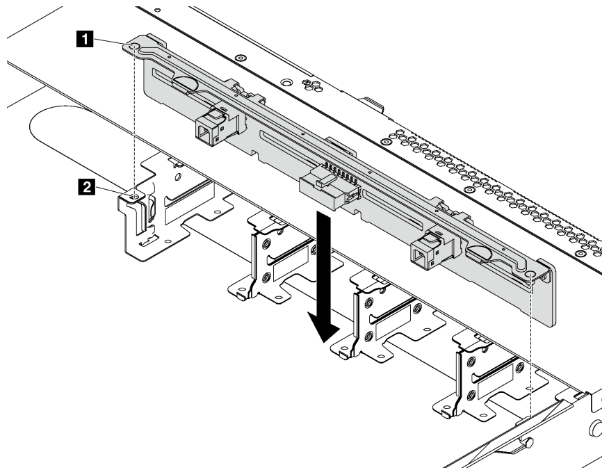
図47. バックプレーンの取り付け
