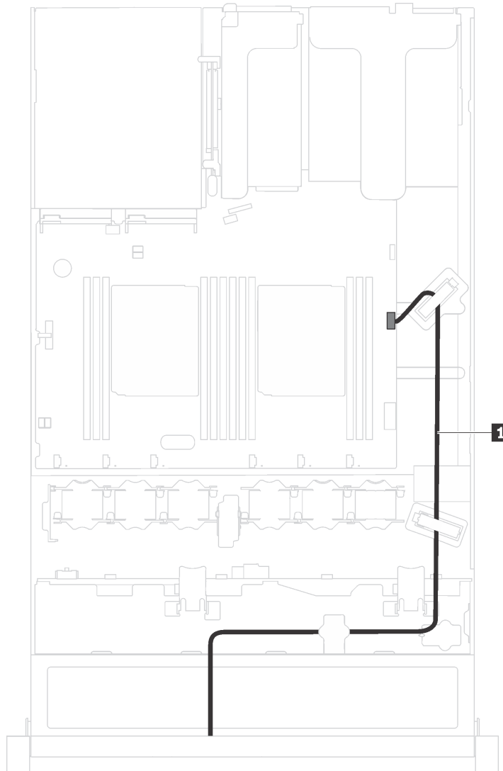
図 13. VGA コネクターのケーブル配線
