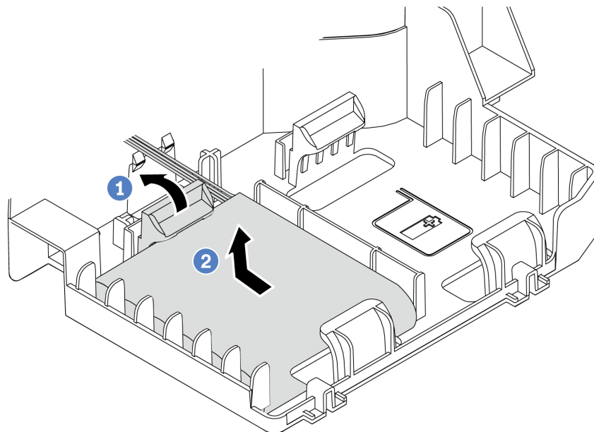
図 36. RAID 超コンデンサー・モジュールの取り外し
