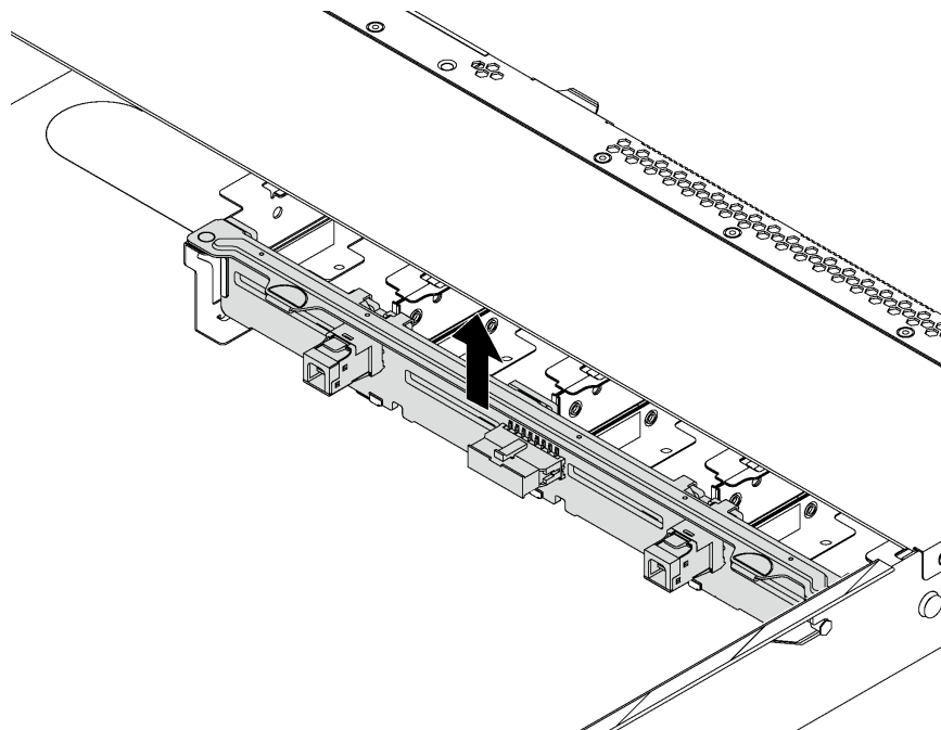
図46. バックプレーンの取り外し
