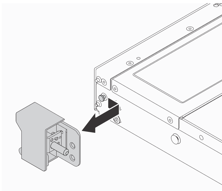
図23. ラック・ラッチの取り外し
