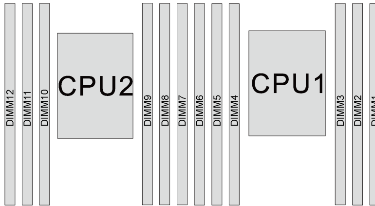
図 57. システム・ボード上のメモリー・モジュール・スロット
