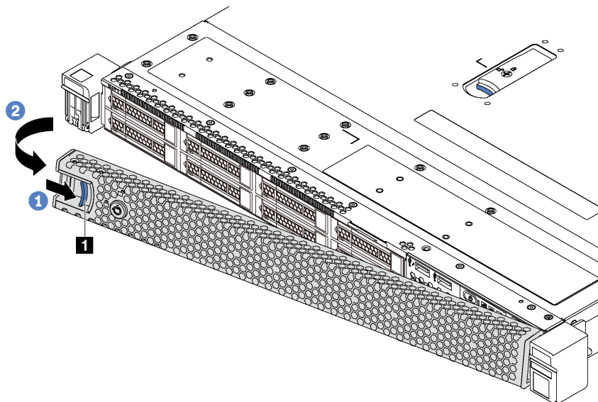
図 28. セキュリティー・ベゼルの取り外し
