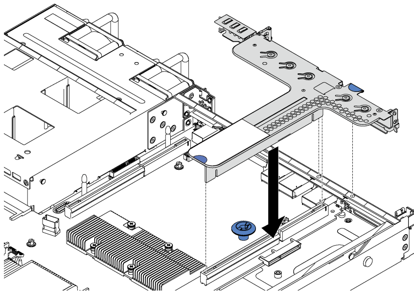
図 79. ライザー・アセンブリーの取り付け
