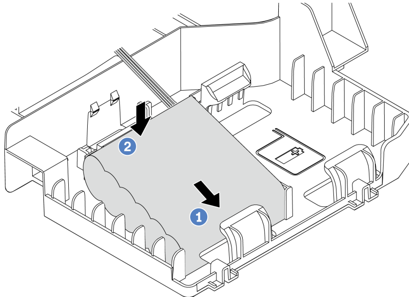
図 37. RAID 超コンデンサー・モジュールの取り付け
