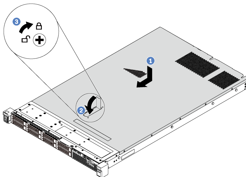
図 33. トップ・カバーの取り付け
