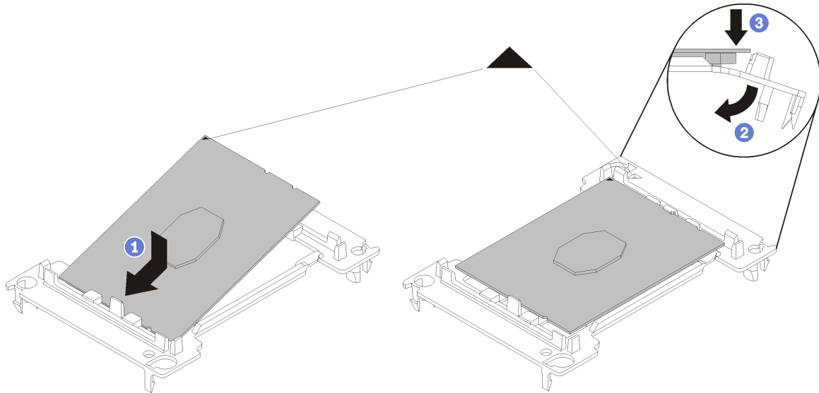
図95. プロセッサ保持器具の取り付け
