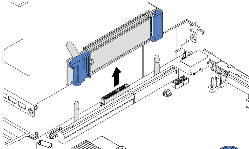
図 80. M.2 バックプレーンの取り外し
