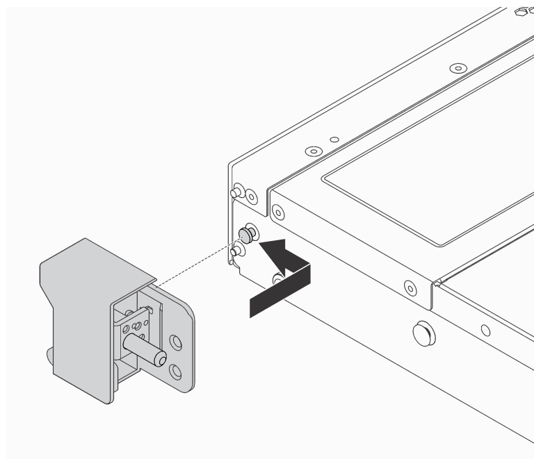
図24. ラック・ラッチの取り付け
