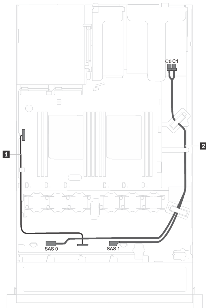
図 17. 8 台の 2.5 型ホット・スワップ・ドライブを搭載したサーバー・モデルのケーブル配線
