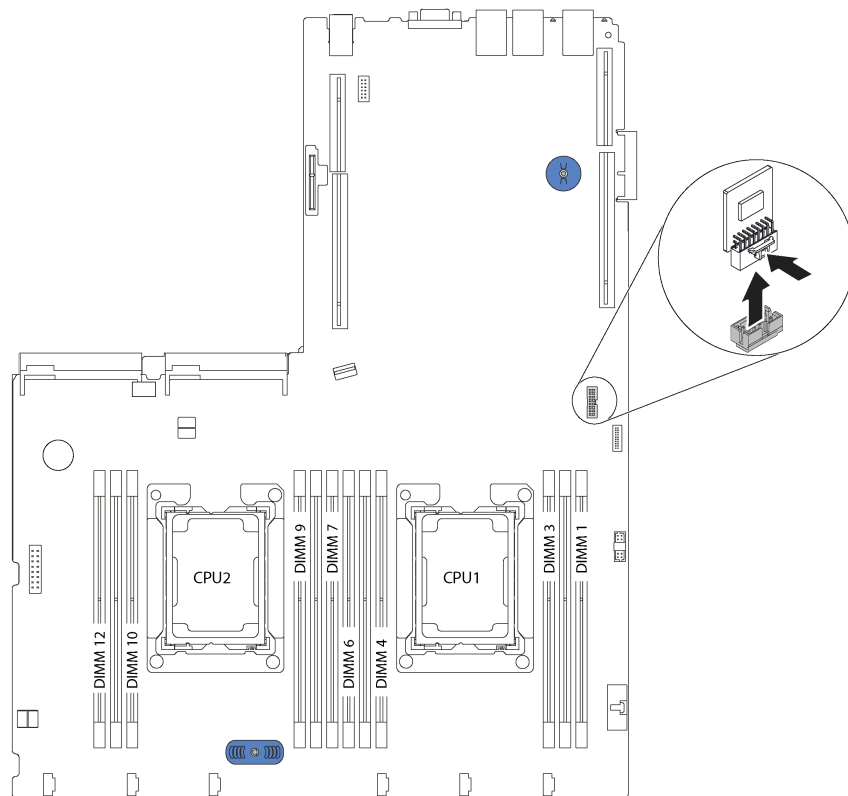
図 61. TCM/TPM アダプターの取り外し
