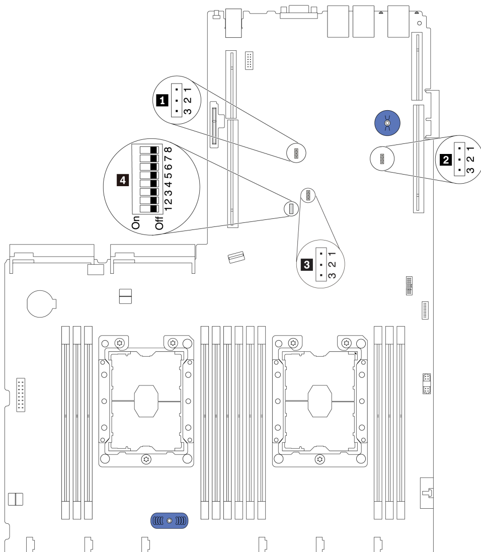
図 11. システム・ボードのスイッチとジャンパー
