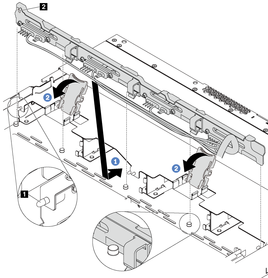
図 49. シンプル・スワップ・ドライブ・バックプレート・アセンブリの取り付け
