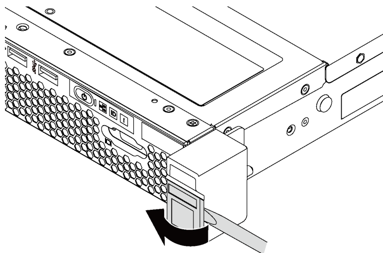
図21. IDラベル・プレートの取り外し
