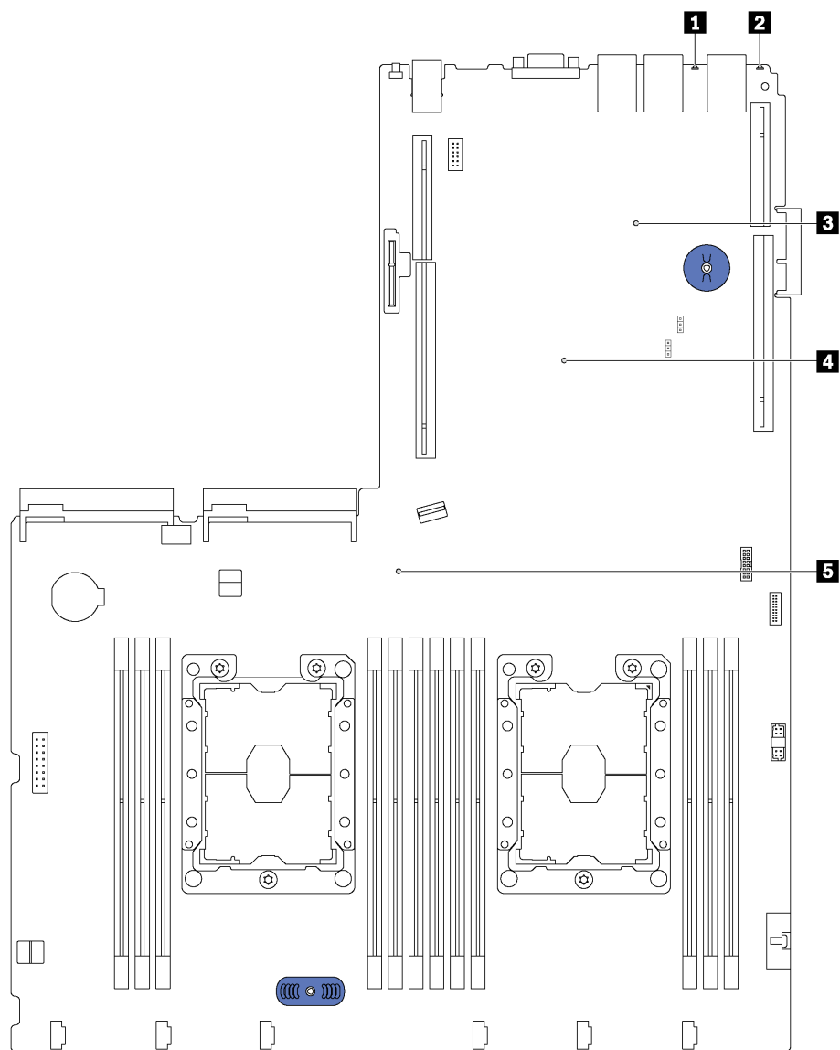
図 12. システム・ボード LED
