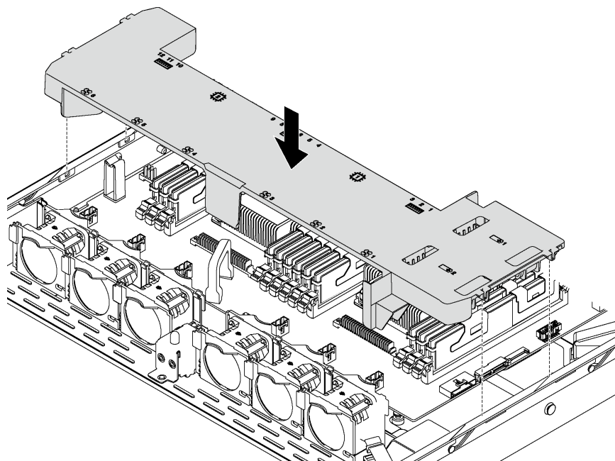
図35. エアー・バッフルの取り付け
