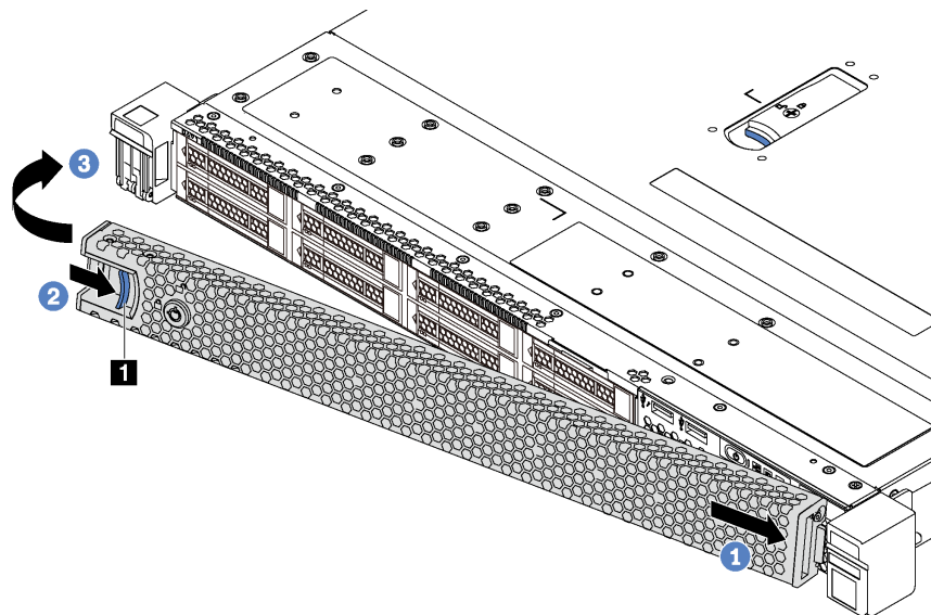
図 30. セキュリティー・ベゼルの取り付け
