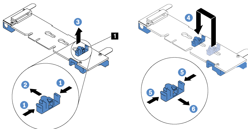
図 82. M.2 保持器具の調整
