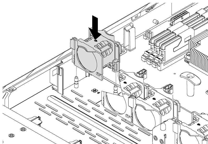
図 39. システム・ファンの取り付け
