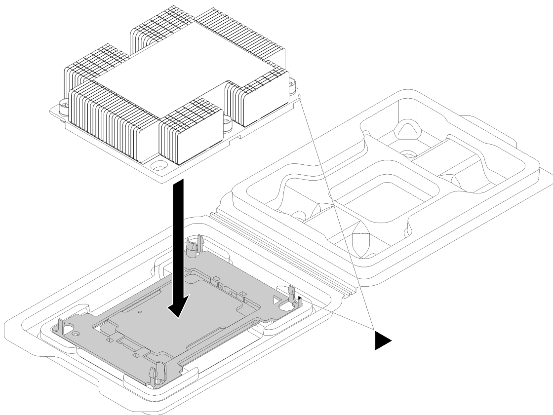
図97. 配送用トレイ内で PHM をアセンブルする
