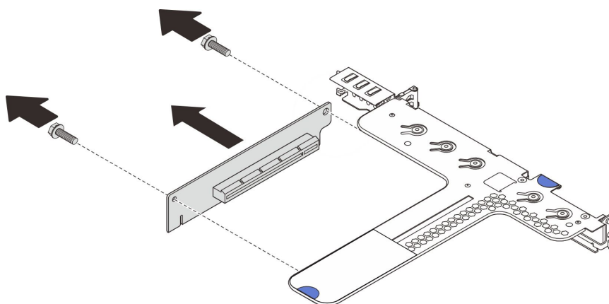
図77. ライザー・カードの取り外し
