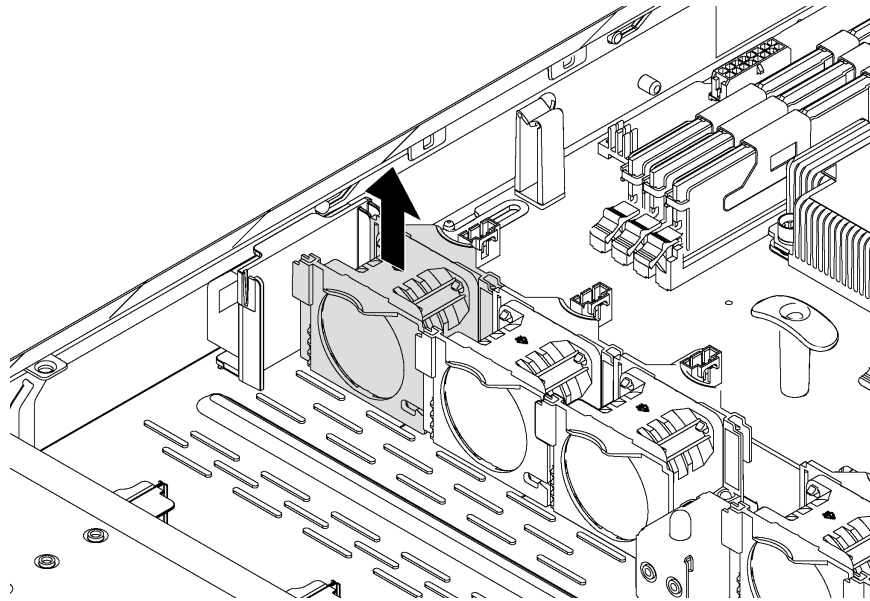
図38. システム・ファンの取り外し
