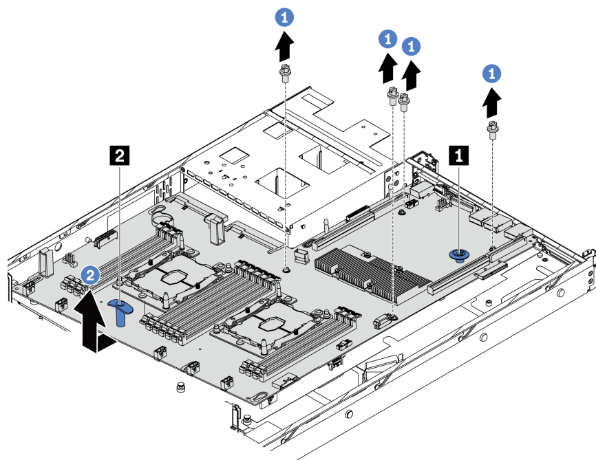
図 99. システム・ボードの取り外し
