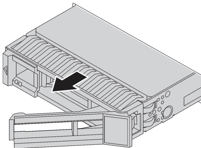
図51. ドライブをドライブ・ベイから引き出す
