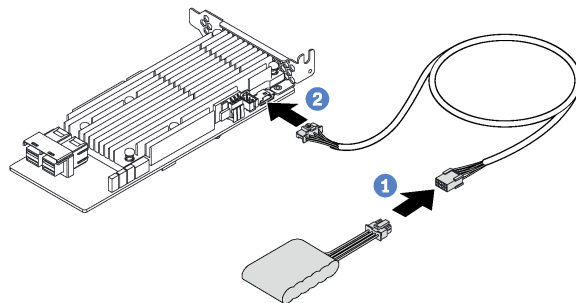
図 16. RAID 超コンデンサー・モジュールの RAID アダプターへの接続
