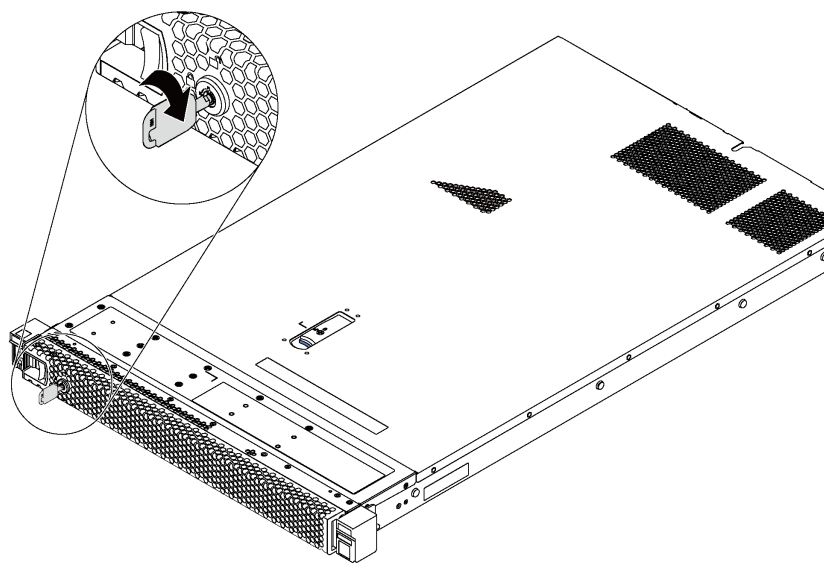
図27. セキュリティー・ベゼルのロック解除
