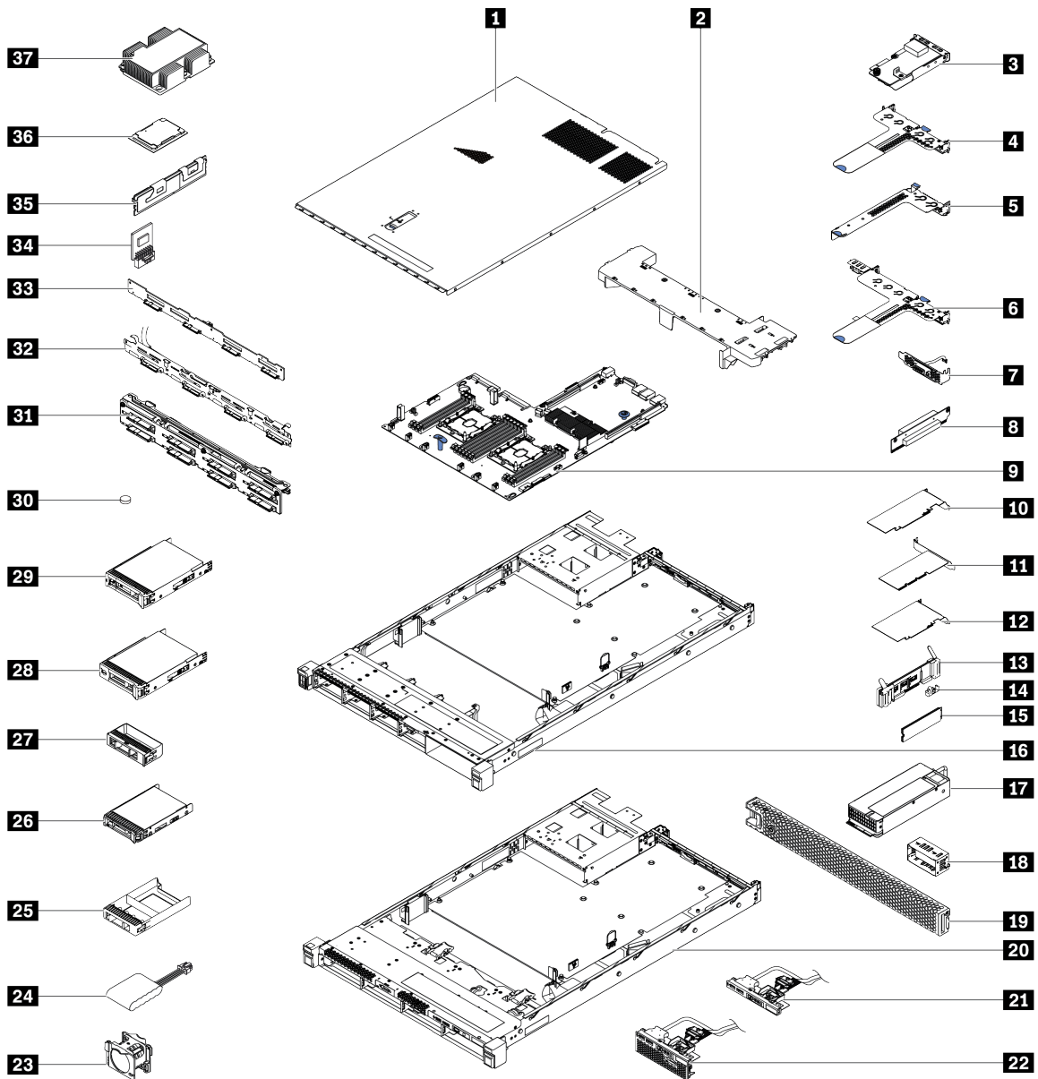
図 20. サーバー・コンポーネント
