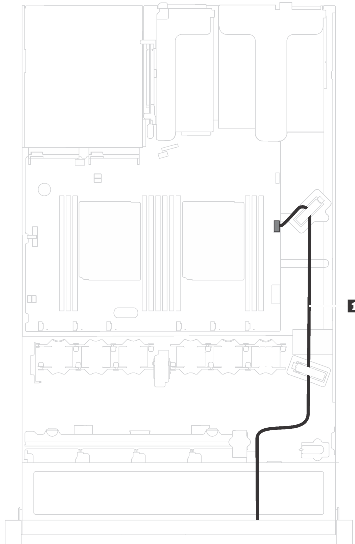
図 14. VGA コネクタのケーブル配線
