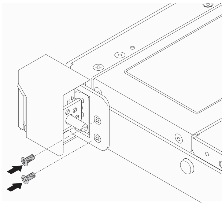
図25. ラック・ラッチのねじの取り付け
