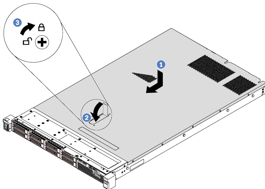
Рис. 33. Установка верхнего кожуха
