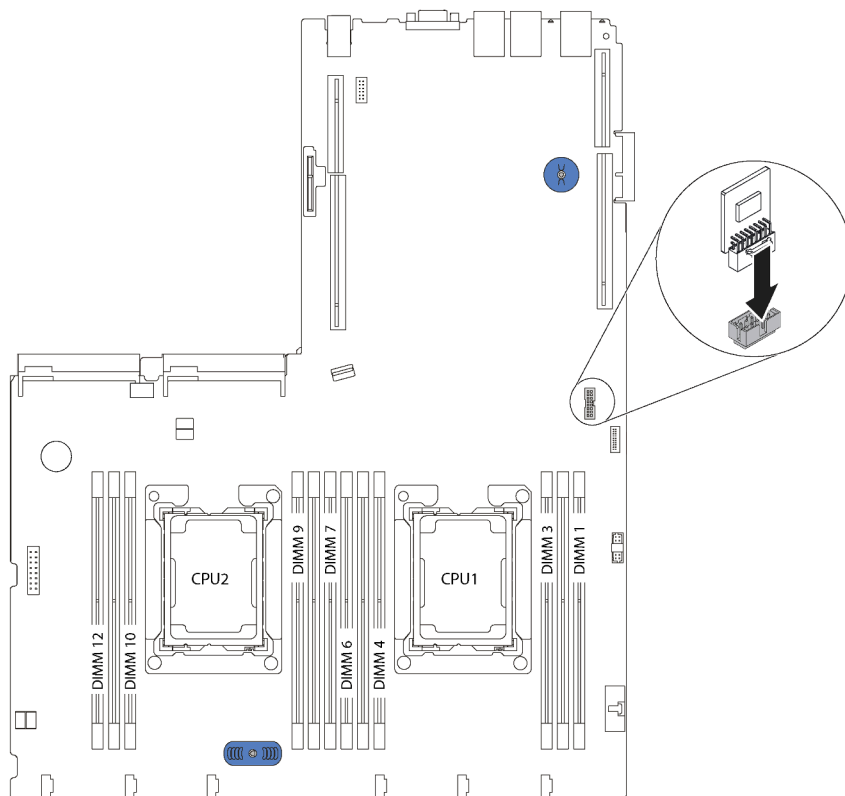
Рис. 62. Установка адаптера TSM/TPM
