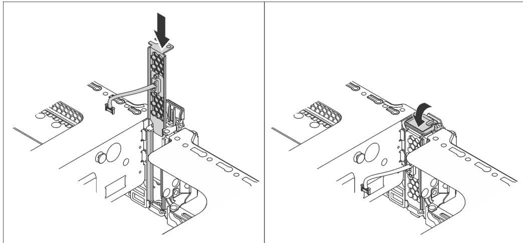
Abbildung 39. Installation des seriellen Anschlussmoduls
