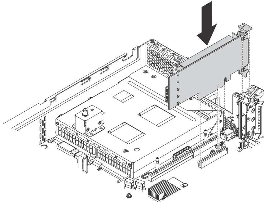
Abbildung 43. PCIe-Adapter auf der Systemplatine installieren
