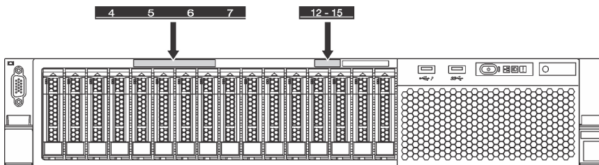
Abbildung 35. Laufwerkpositionsetiketten für Servermodelle, auf denen zwei SATA/SAS-Rückwandplatten installiert sind
