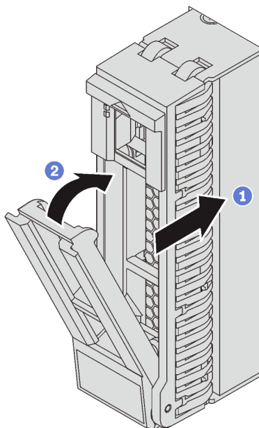
Abbildung 58. Installation eines 2,5-Zoll-Hot-Swap-Laufwerks
