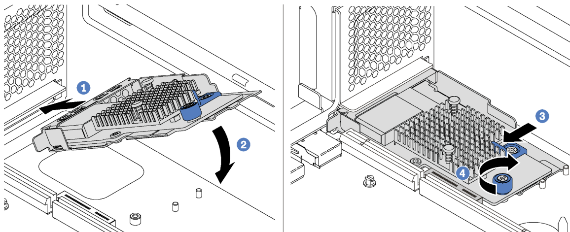
Abbildung 40. Installieren eines LOM-Adapters
