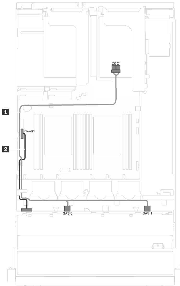
Abbildung 17. Kabelführung für Servermodelle mit acht 3,5-Zoll-Hot-Swap-Laufwerken und seriellem Anschlussmodul
