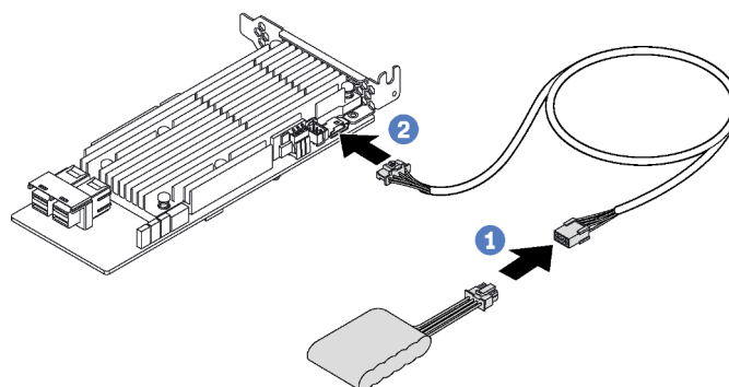
Abbildung 54. Anschließen des RAID-Superkondensatormoduls am RAID-Adapter
