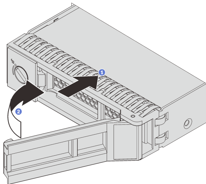
Abbildung 61. Installation eines Simple-Swap-Laufwerks
