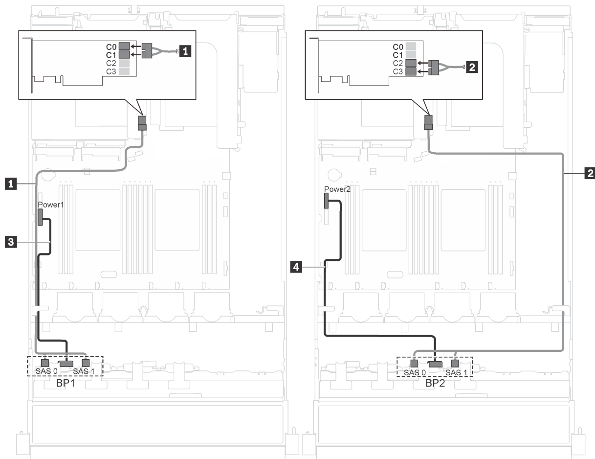
Abbildung 24. Kabelführung für Servermodelle mit sechzehn 2,5-Zoll-Hot-Swap-Laufwerken und 16i-Adapter
