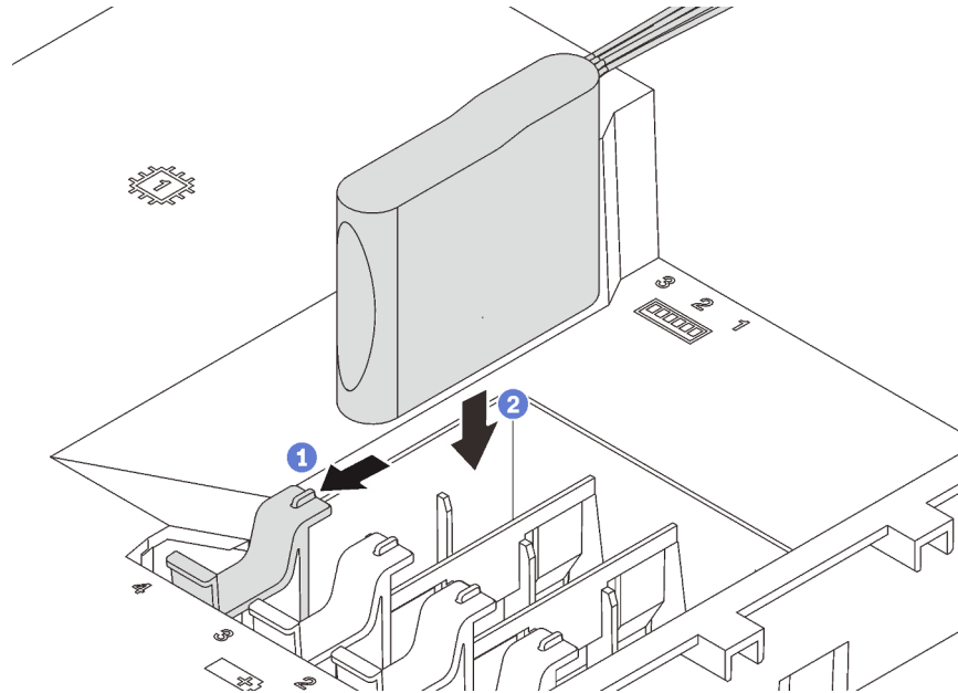
Abbildung 53. Installation des RAID-Superkondensatormoduls
