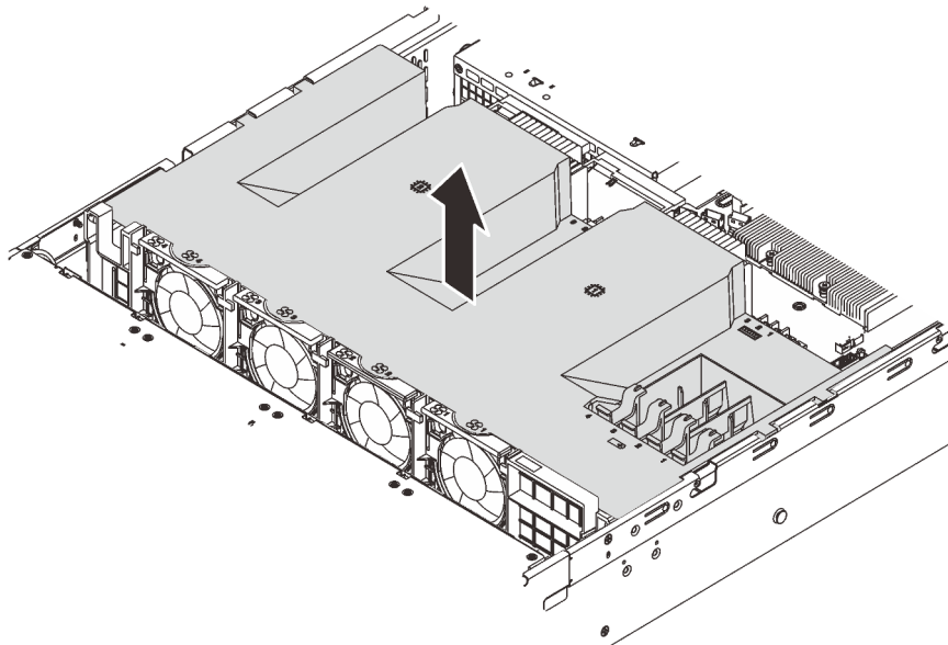
Abbildung 30. Entfernen der Luftführung
