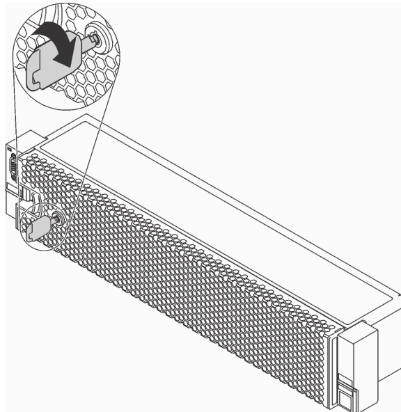
Abbildung 27. Sicherheitsfrontblende aufschließen
