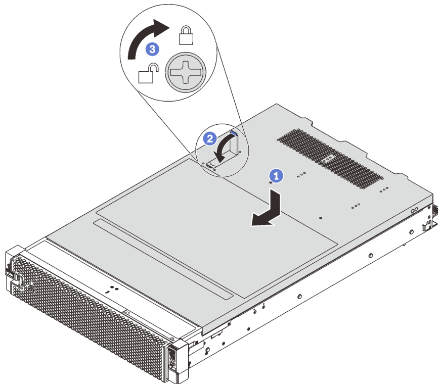
Abbildung 55. Installation der oberen Abdeckung
