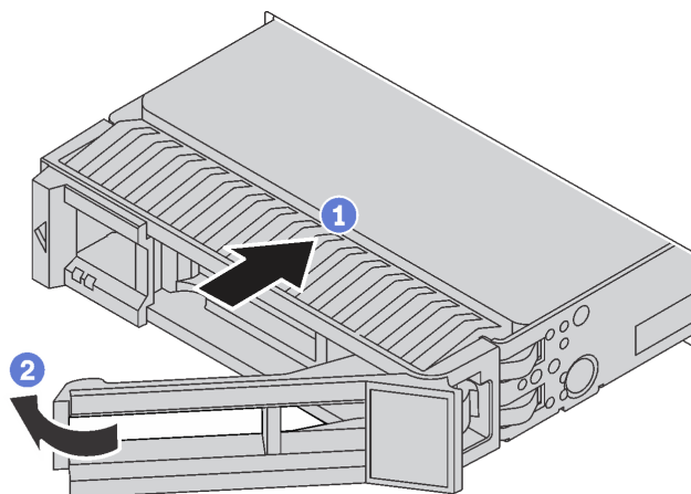
Abbildung 59. Installation eines 3,5-Zoll-Hot-Swap-Laufwerks
