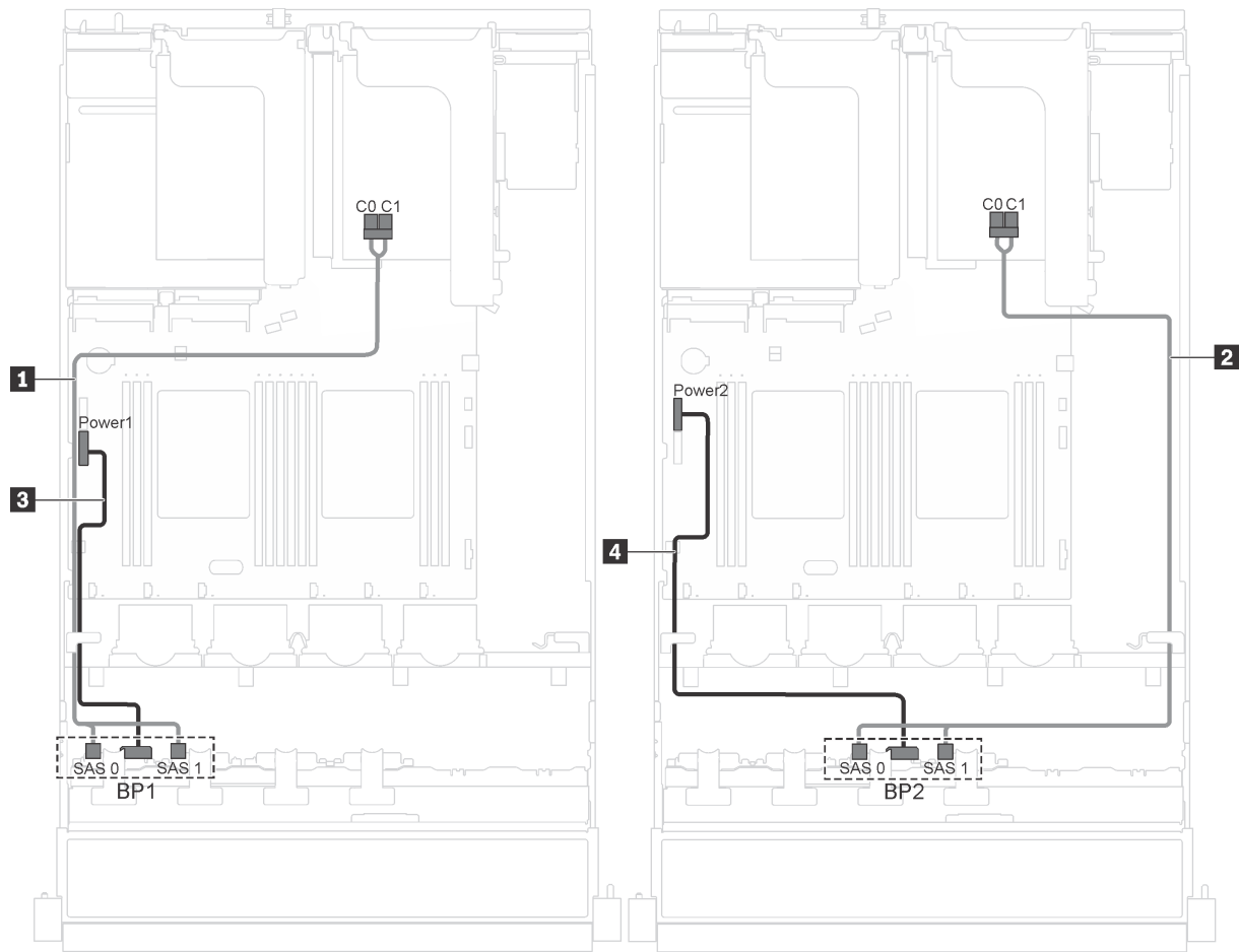
Abbildung 23. Kabelführung für Servermodelle mit sechzehn 2,5-Zoll-Hot-Swap-Laufwerken, 8i-Adaptoren und seriellen Anschlussmodul
