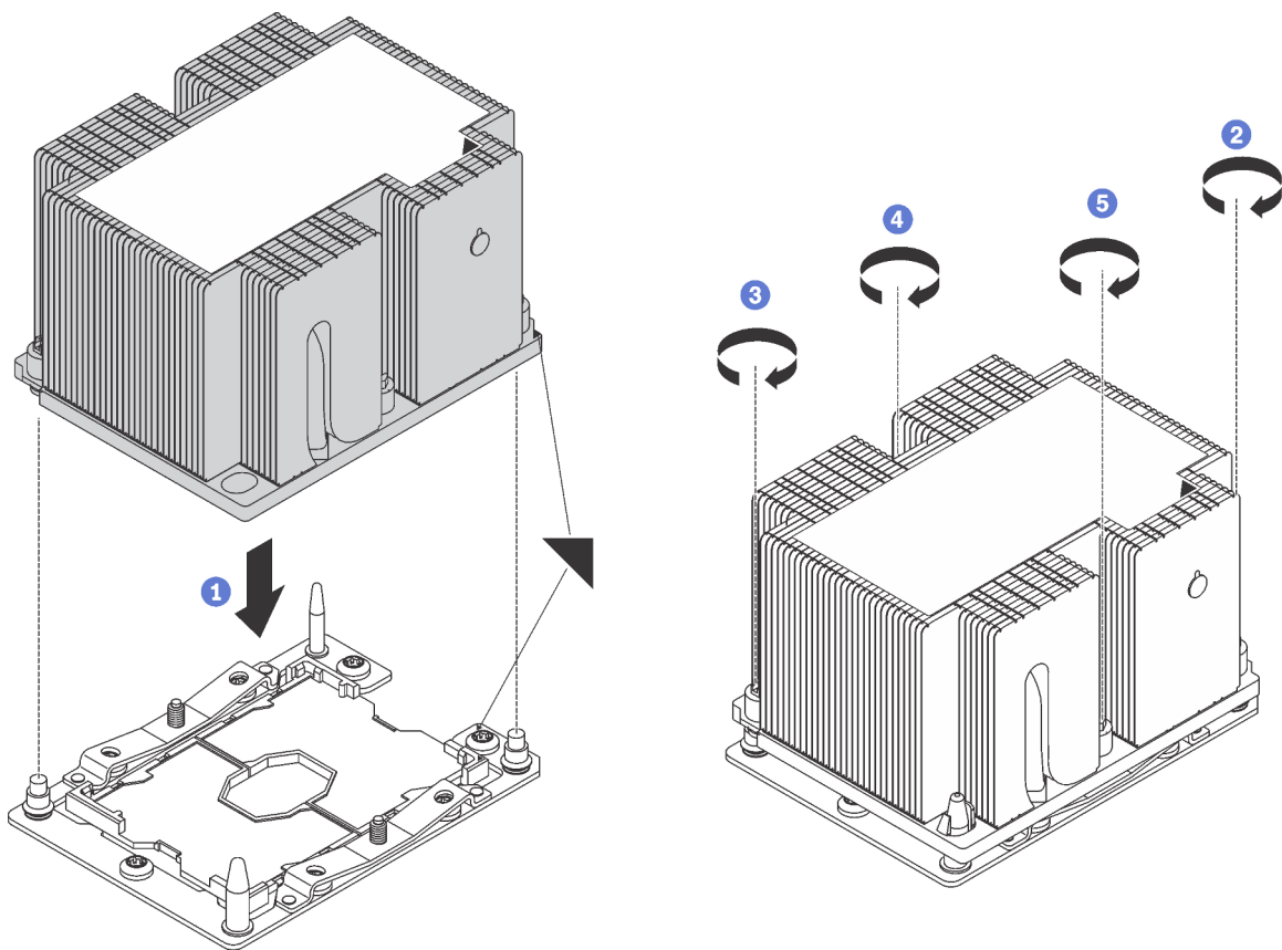
Abbildung 31. Installieren des PHM
