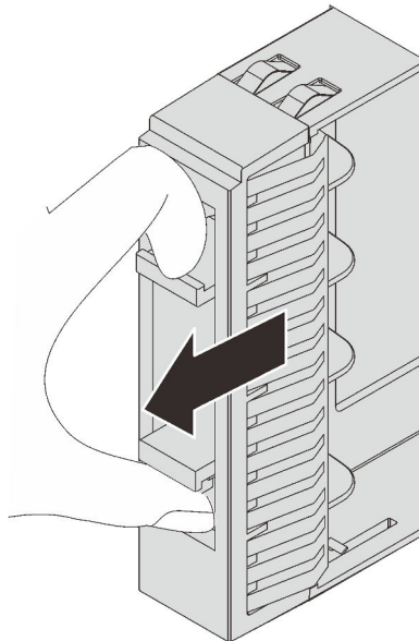
Abbildung 56. Entfernen der Abdeckblende für 2,5-Zoll-Laufwerke
