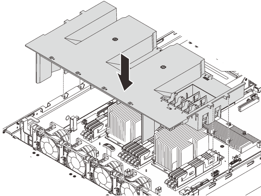
Abbildung 52. Installation der Luftführung
