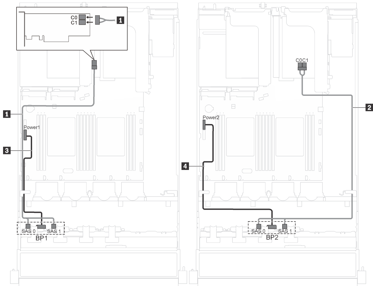
Abbildung 22. Kabelführung für Servermodelle mit sechzehn 2,5-Zoll-Hot-Swap-Laufwerken und zwei 8i Adaptern
