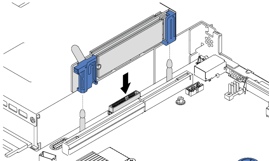
Abbildung 46. Installieren der M.2-Rückwandplatine
