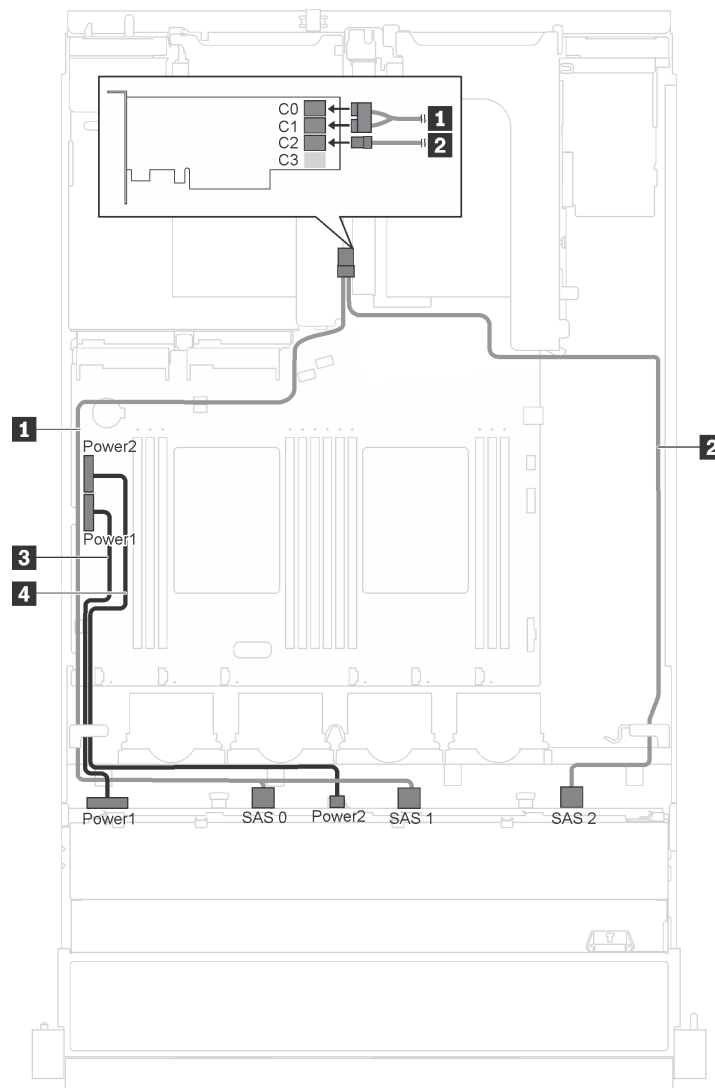
Abbildung 18. Kabelführung für Servermodelle mit zwölf 3,5-Zoll-Hot-Swap-Laufwerken und 16i-Adapter
