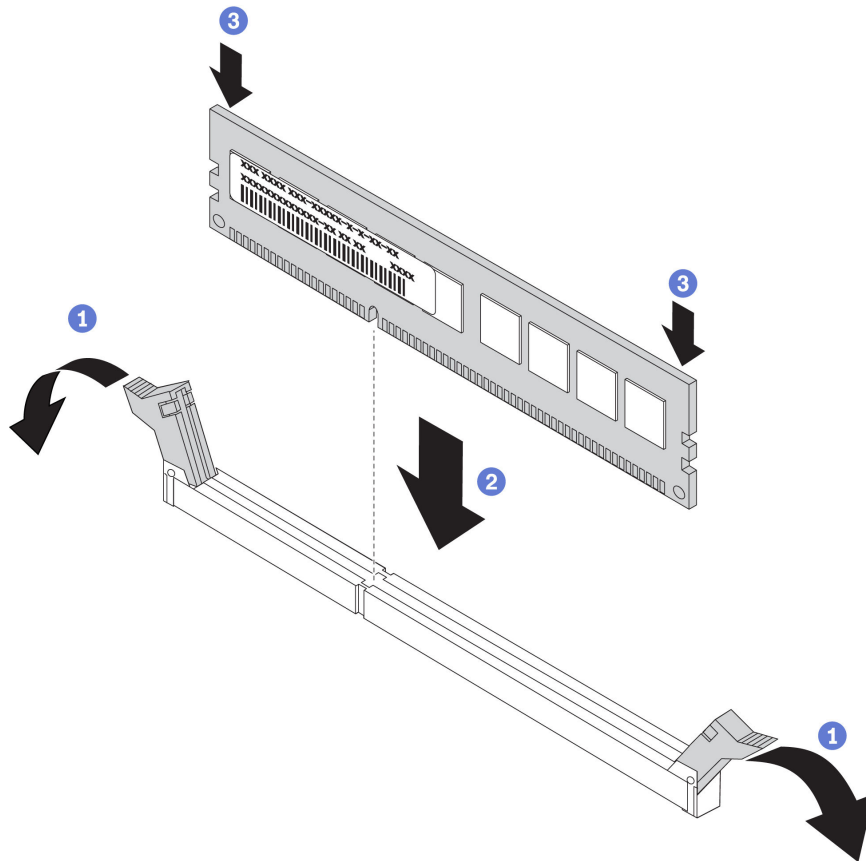
Abbildung 32. Speichermodul installieren
