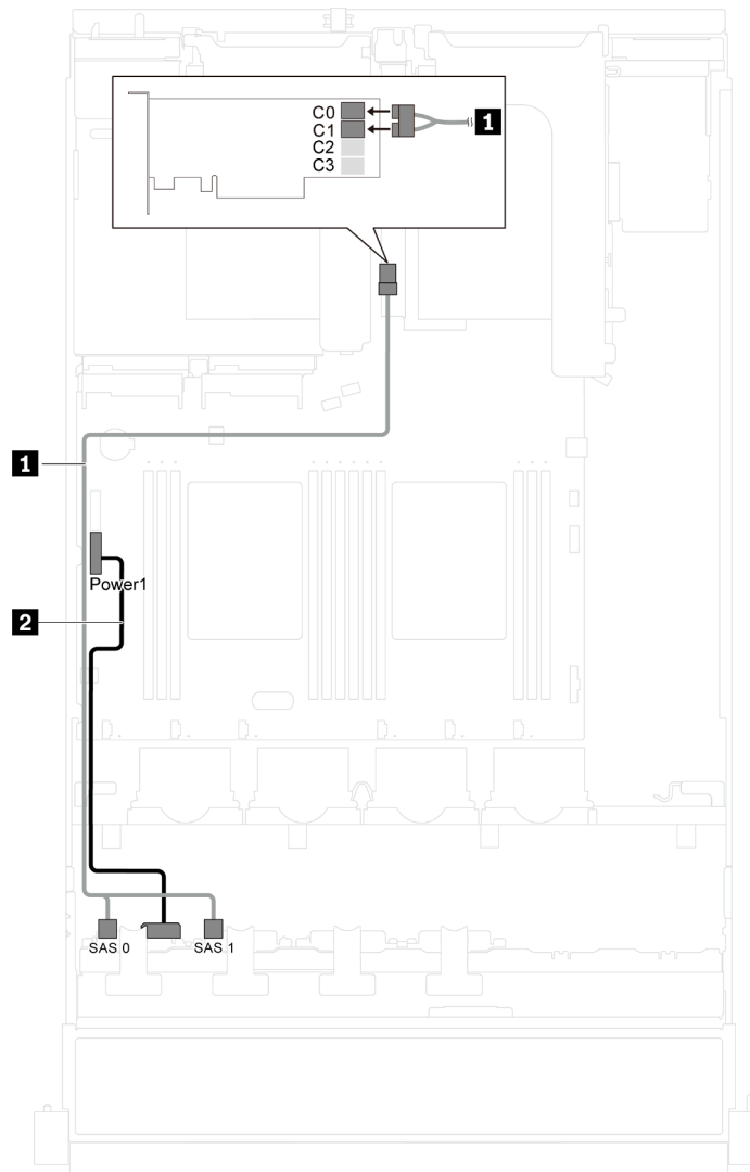
Abbildung 20. Kabelführung für Servermodelle mit acht 2,5-Zoll-Hot-Swap-Laufwerken
