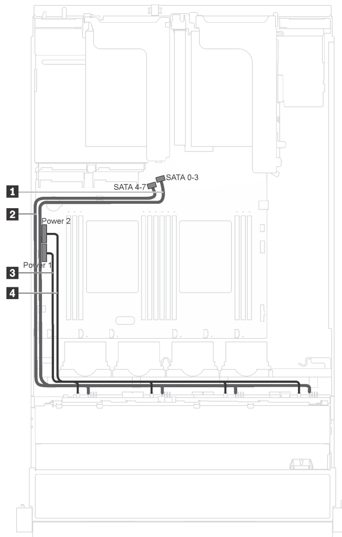
Abbildung 15. Kabelführung für Servermodelle mit acht 3,5-Zoll-Simple-Swap-Laufwerken
