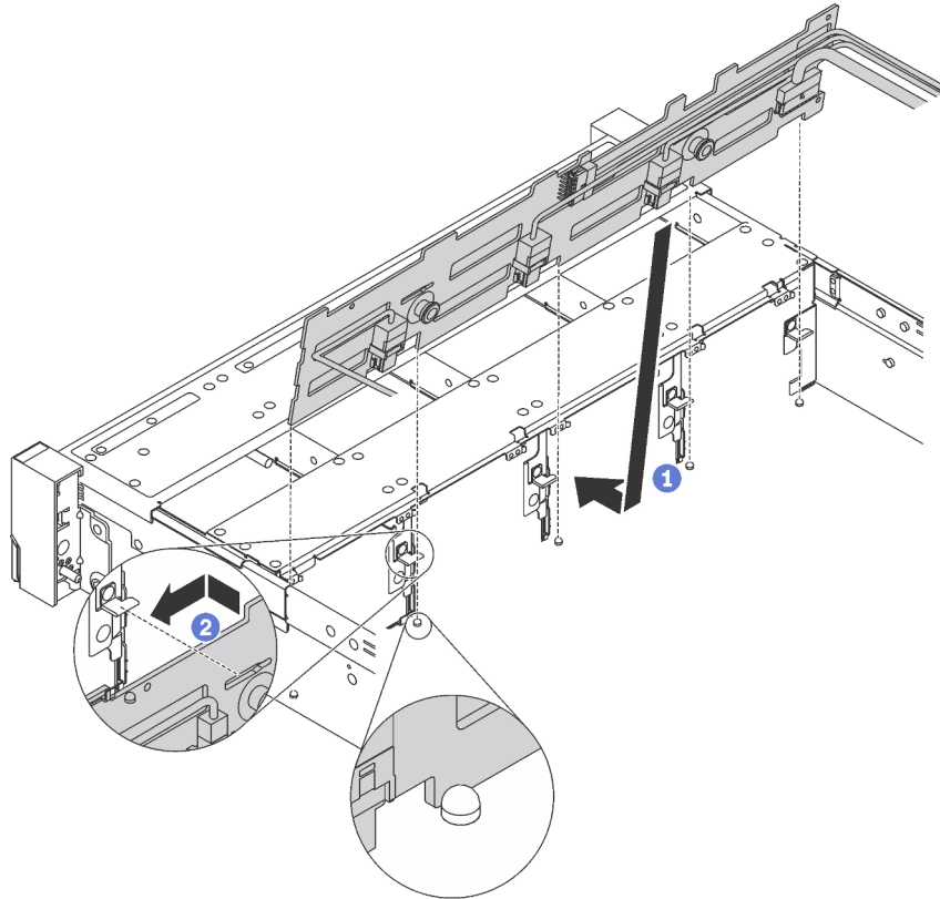
Abbildung 36. Installation der Rückwandplatte für 3,5"-Laufwerke
