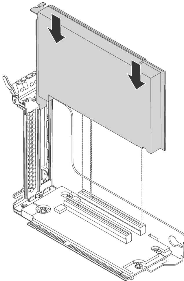
Abbildung 41. Installieren eines PCIe-Adapters auf der Adapterkartenbaugruppe
