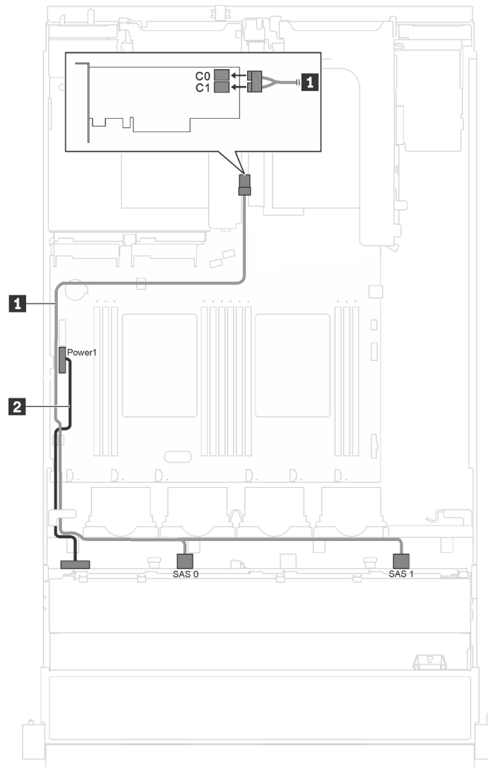
Abbildung 16. Kabelführung für Servermodelle mit acht 3,5-Zoll-Hot-Swap-Laufwerken
