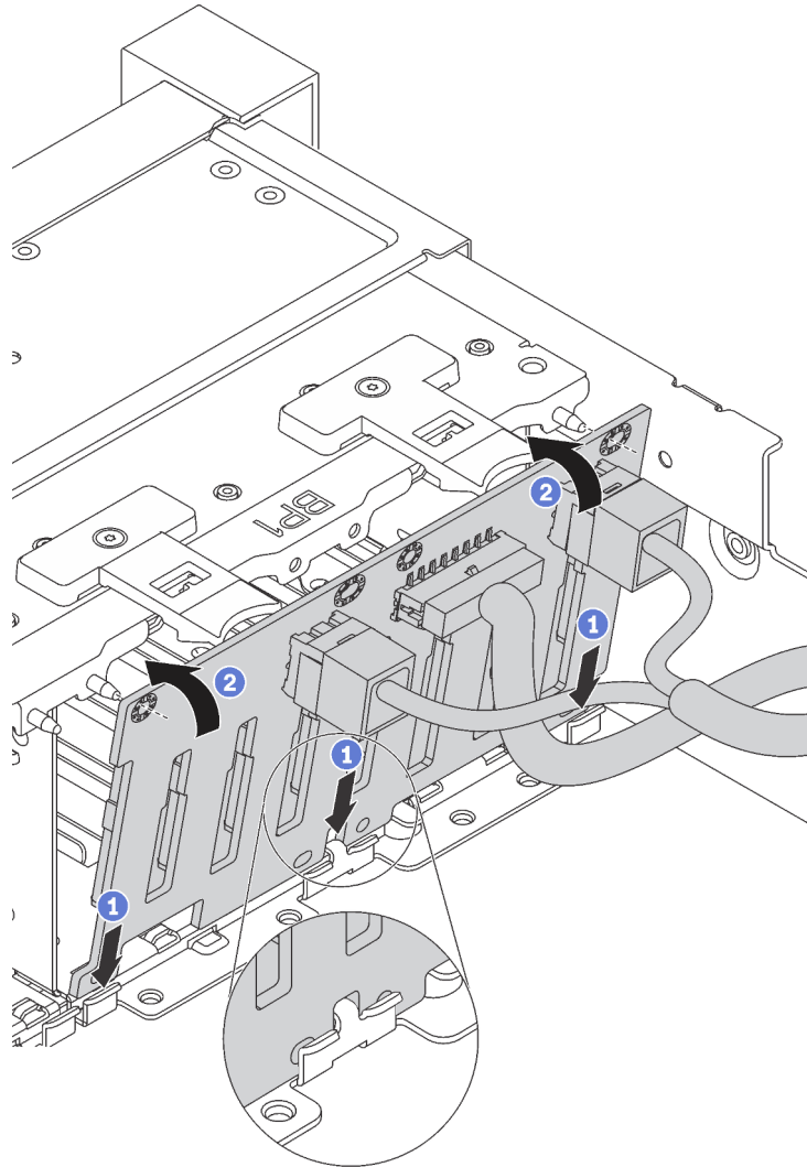
Abbildung 34. Installation der Rückwandplatine für 2,5-Zoll-Laufwerke
