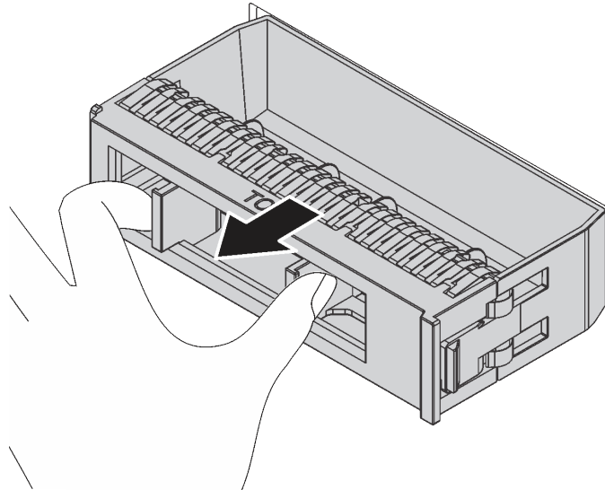
Abbildung 57. Entfernen der Abdeckblende für 3,5-Zoll-Laufwerke
