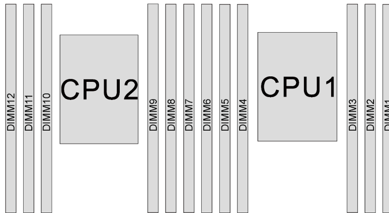
Abbildung 33. Speichermodul-Steckplätze auf der Systemplatine
