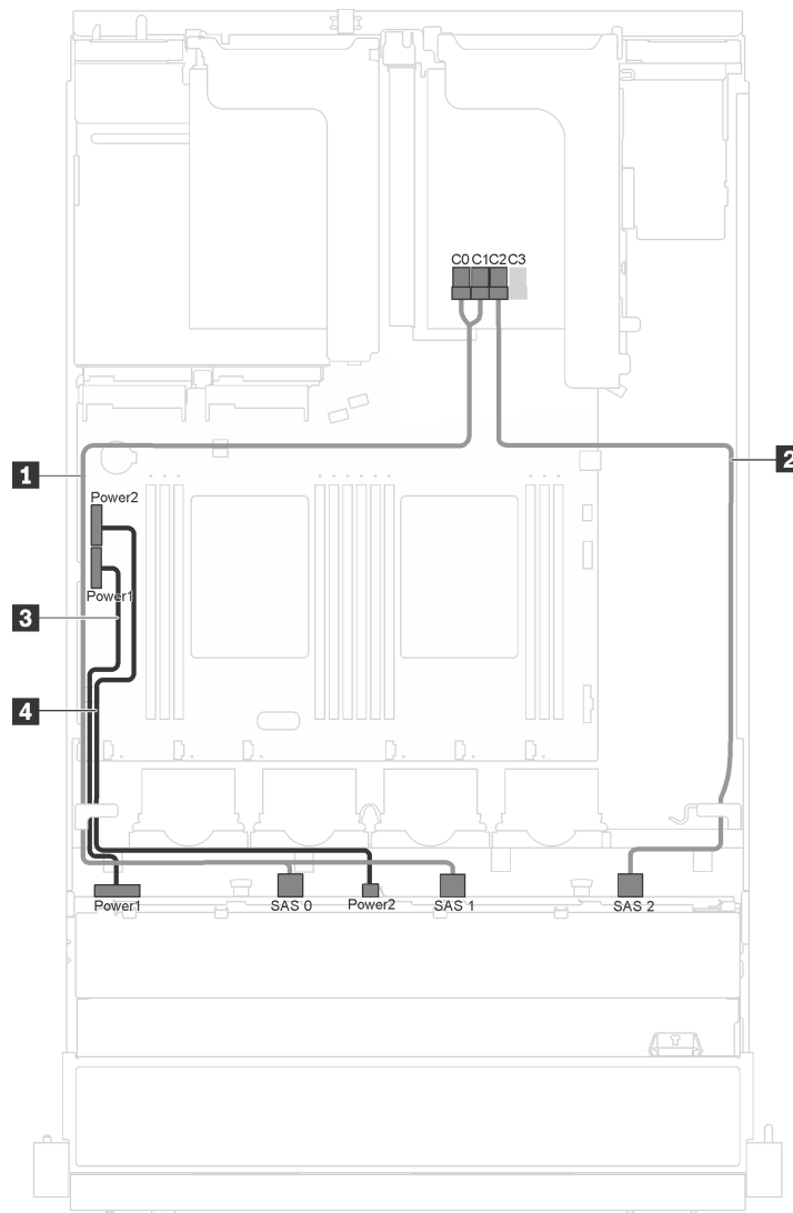
Abbildung 19. Kabelführung für Servermodelle mit zwölf 3,5-Zoll-Hot-Swap-Laufwerken, 16i-Adapter und seriellem Anschlussmodul
