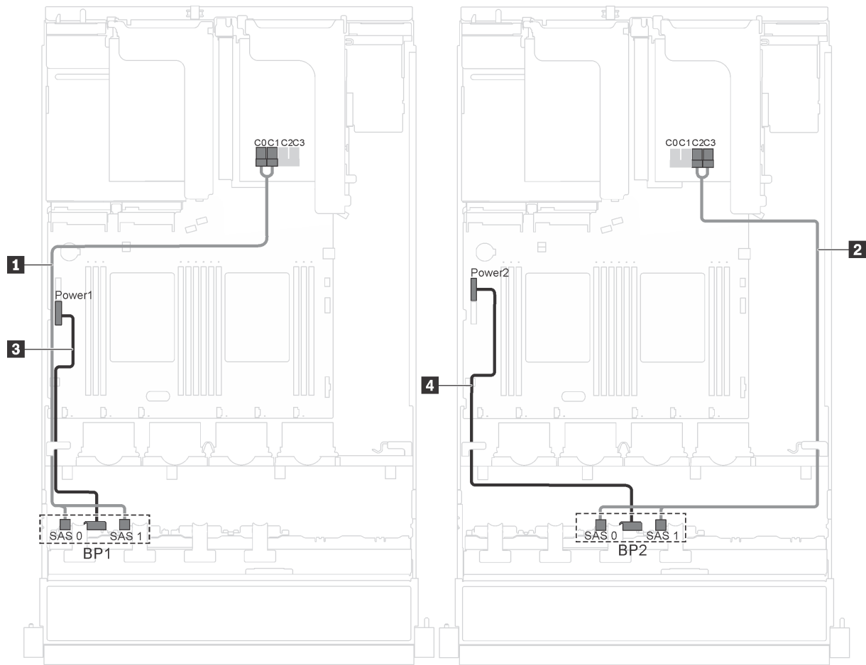
Abbildung 25. Kabelführung für Servermodelle mit sechzehn 2,5-Zoll-Hot-Swap-Laufwerken, 16i-Adapter und seriellm Anschlussmodul
