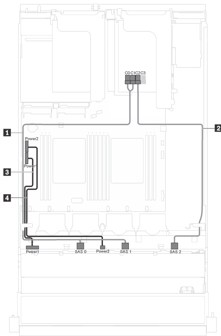
Figura 21. Roteamento de cabos para modelos de servidor com doze unidades hot-swap de 3,5 polegadas, adaptador 16i e módulo de porta serial
