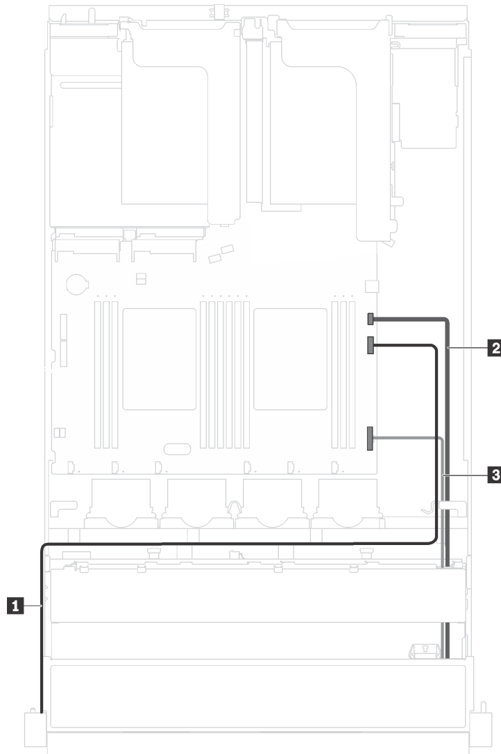
Figura 66. Conexão de cabos do conjunto de E/S frontal
