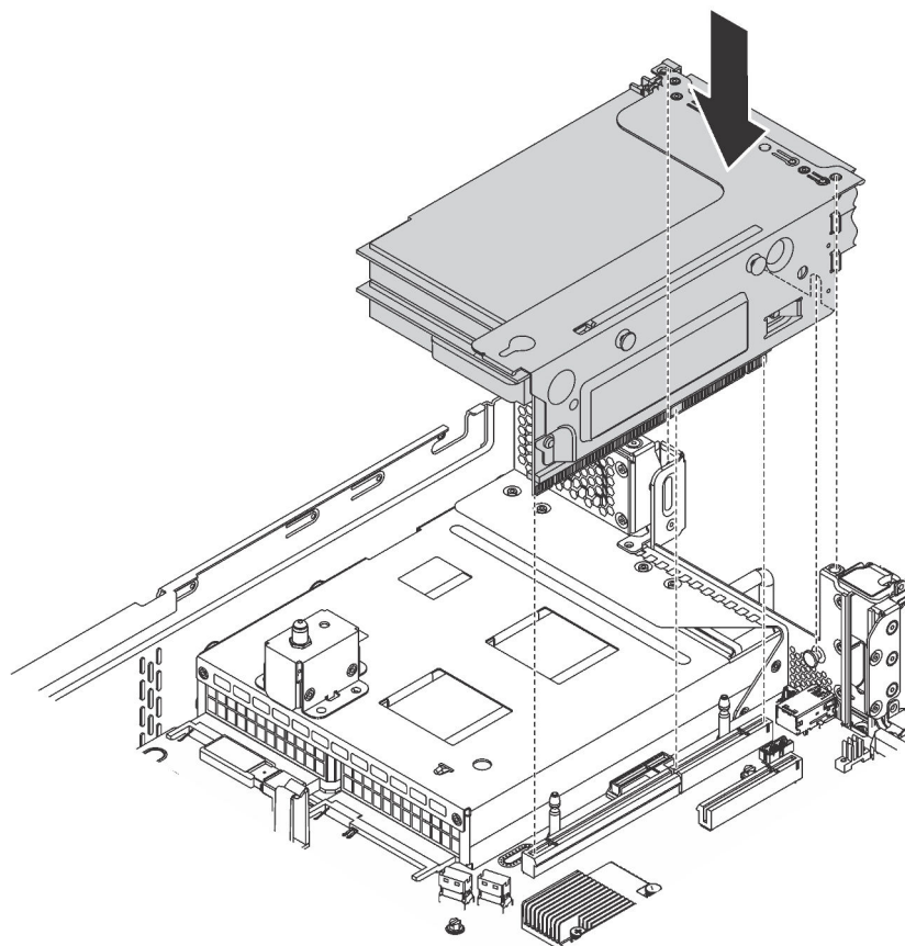
Figura 86. Instalação do conjunto de placa riser 2
