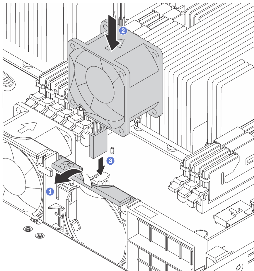
Figura 96. Instalação do ventilador do sistema
