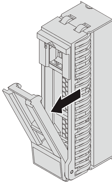
Figura 50. Remoção de uma unidade hot-swap de 2,5 polegadas
