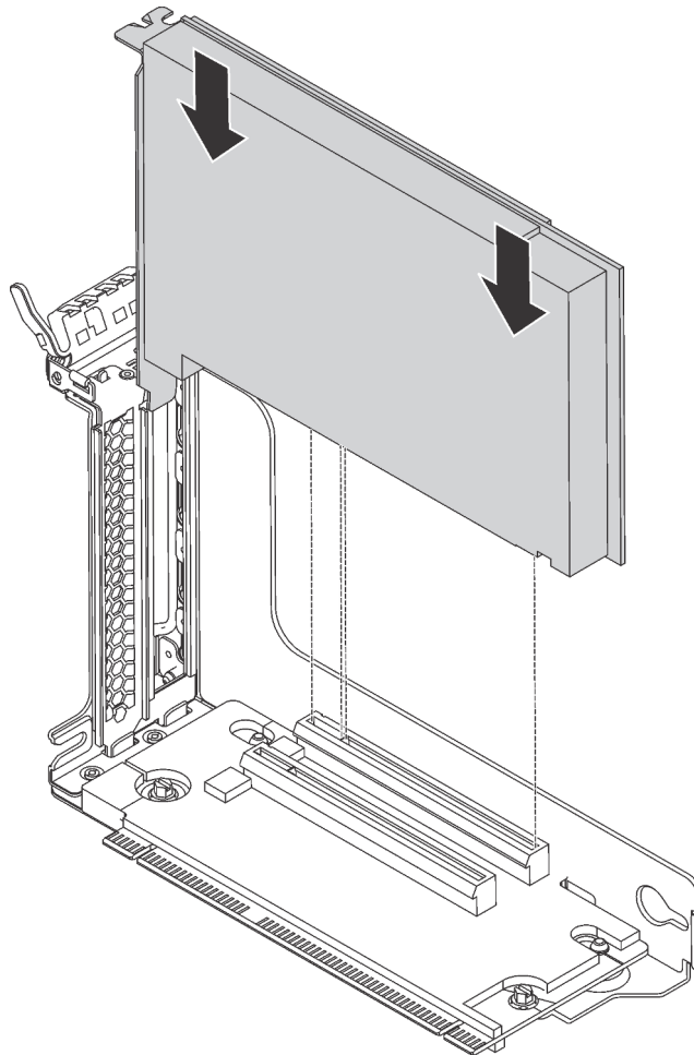
Figura 91. Instalando um adaptador PCIe no conjunto de placa riser
