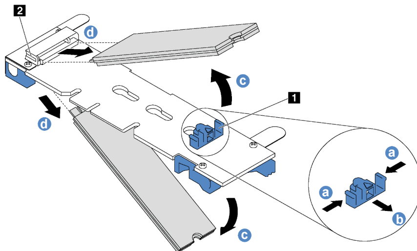
Figura 106. Remoção da unidade M.2
