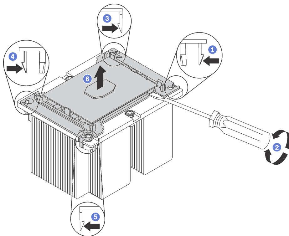
Figura 115. Separando um dissipador de calor de um processador
