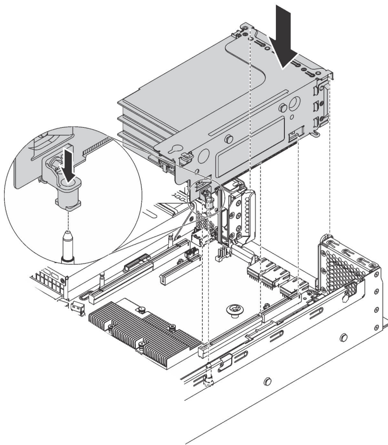
Figura 85. Instalação do conjunto de placa riser 1
