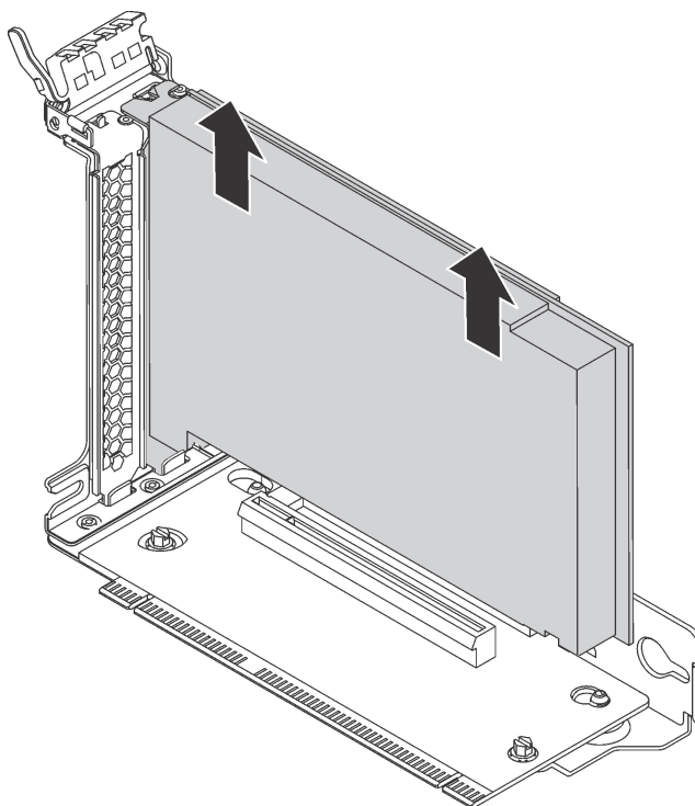
Figura 88. Removendo um adaptador PCIe do conjunto de placa riser
