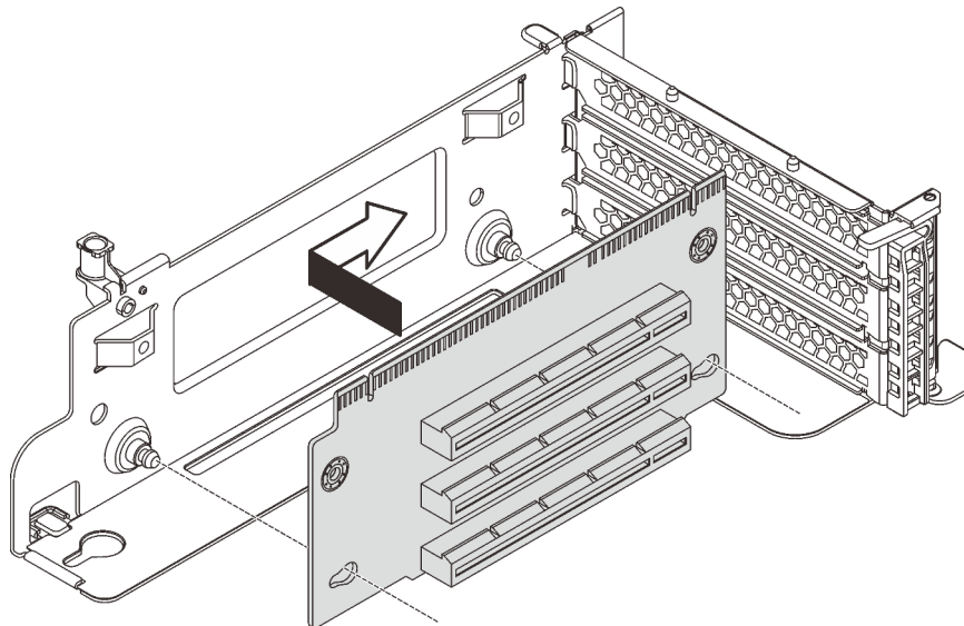
Figura 83. Instalação da placa riser
