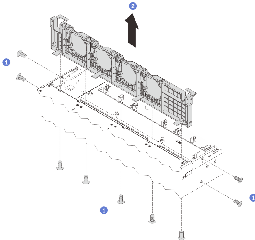
Figura 97. Remoção do compartimento do ventilador do sistema
