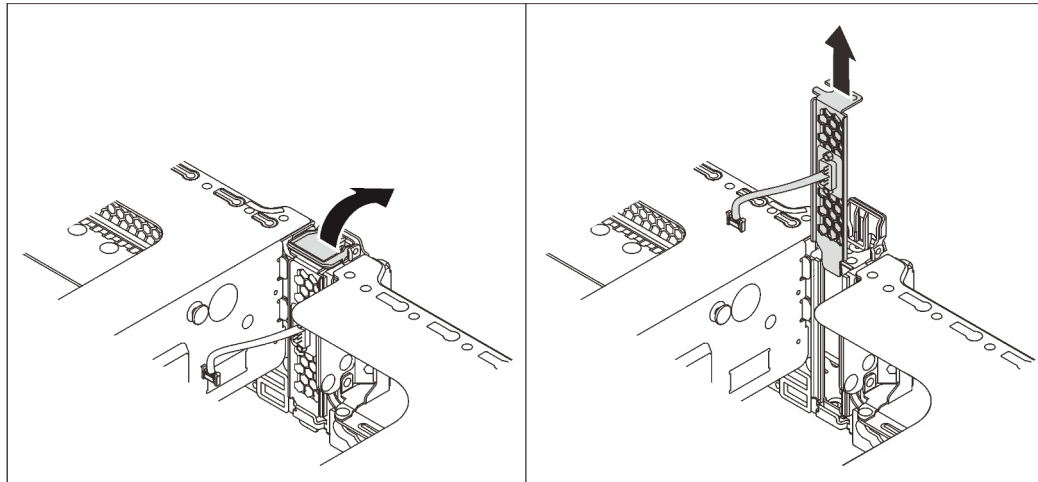
Figura 93. Remoção do módulo de porta serial
