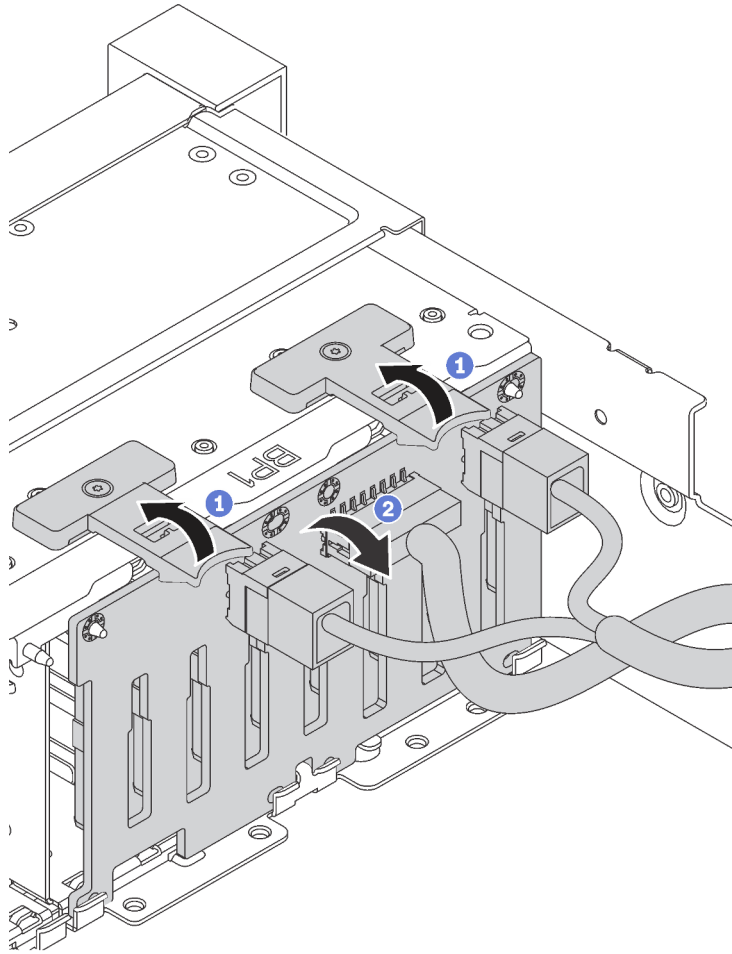
Figura 62. Remoção do painel traseiro da unidade de 2,5 polegadas
