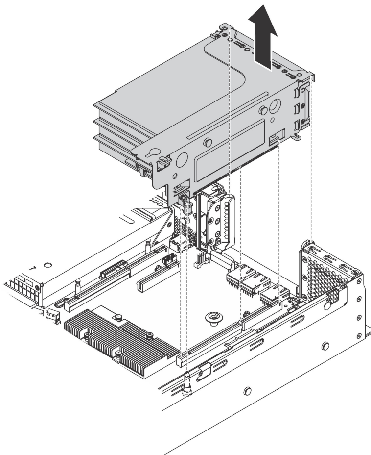
Figura 80. Remoção do conjunto da placa riser 1
