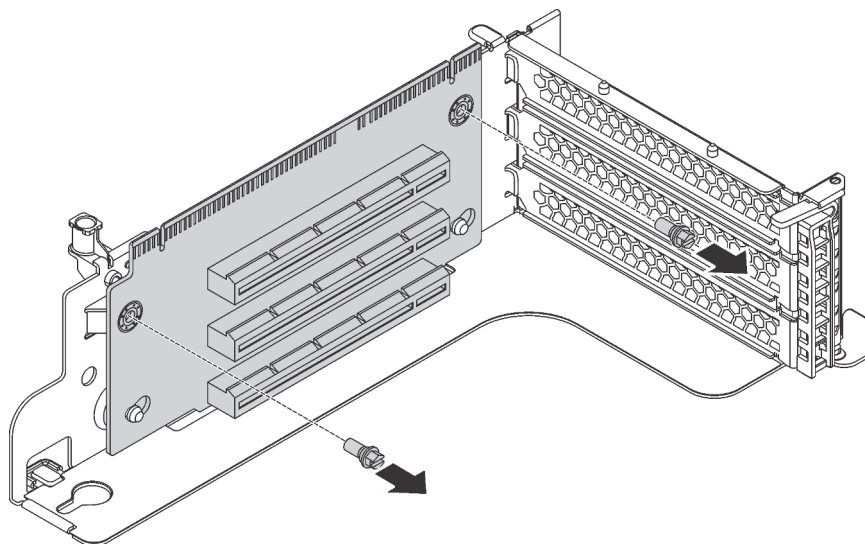
Figura 82. remoção da placa riser
