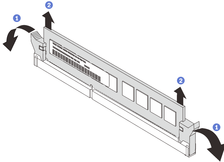
Figura 99. Remoção do módulo de memória
