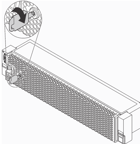
Figura 33. Destravando o painel de segurança
