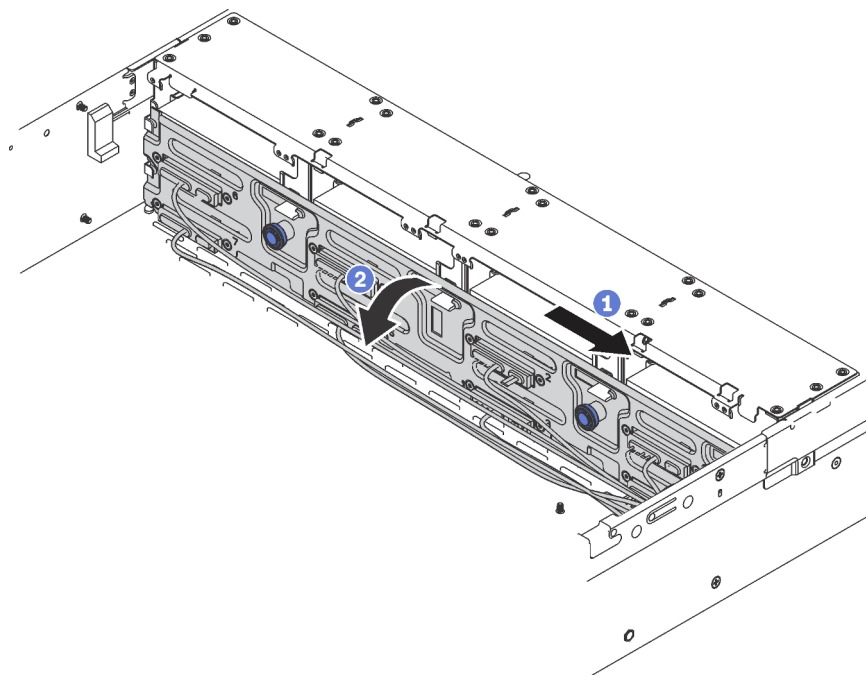
Figura 64. Remoção do conjunto de placa traseira de unidade simple-swap de 3,5 polegadas
