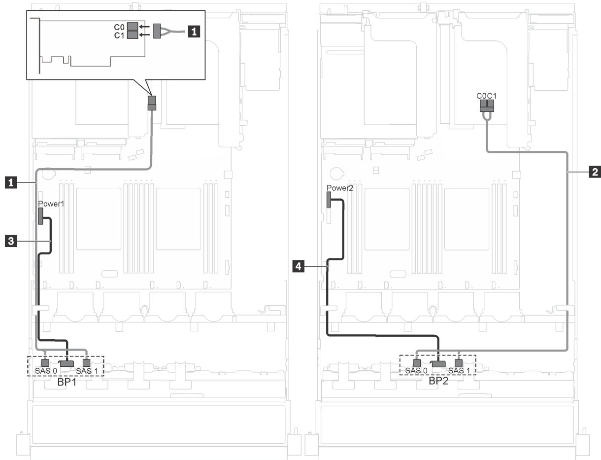
Figura 24. Roteamento de cabos para modelos de servidor com dezesseis unidades hot-swap de 2,5 polegadas e dois adaptadores 8i
