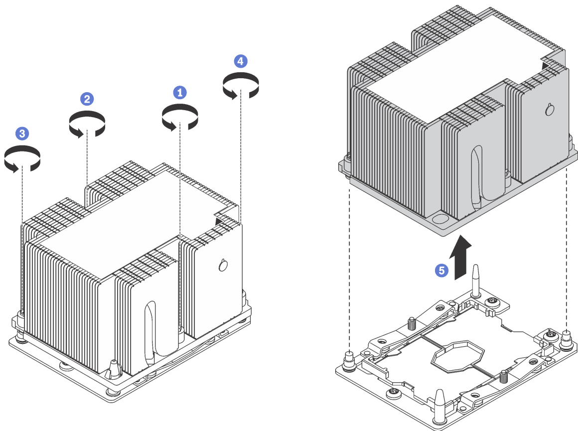
Figura 114. Removendo um PHM
