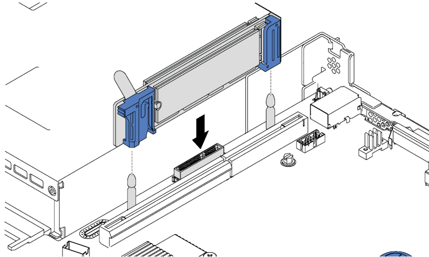
Figura 109. Instalação do backplane M.2
