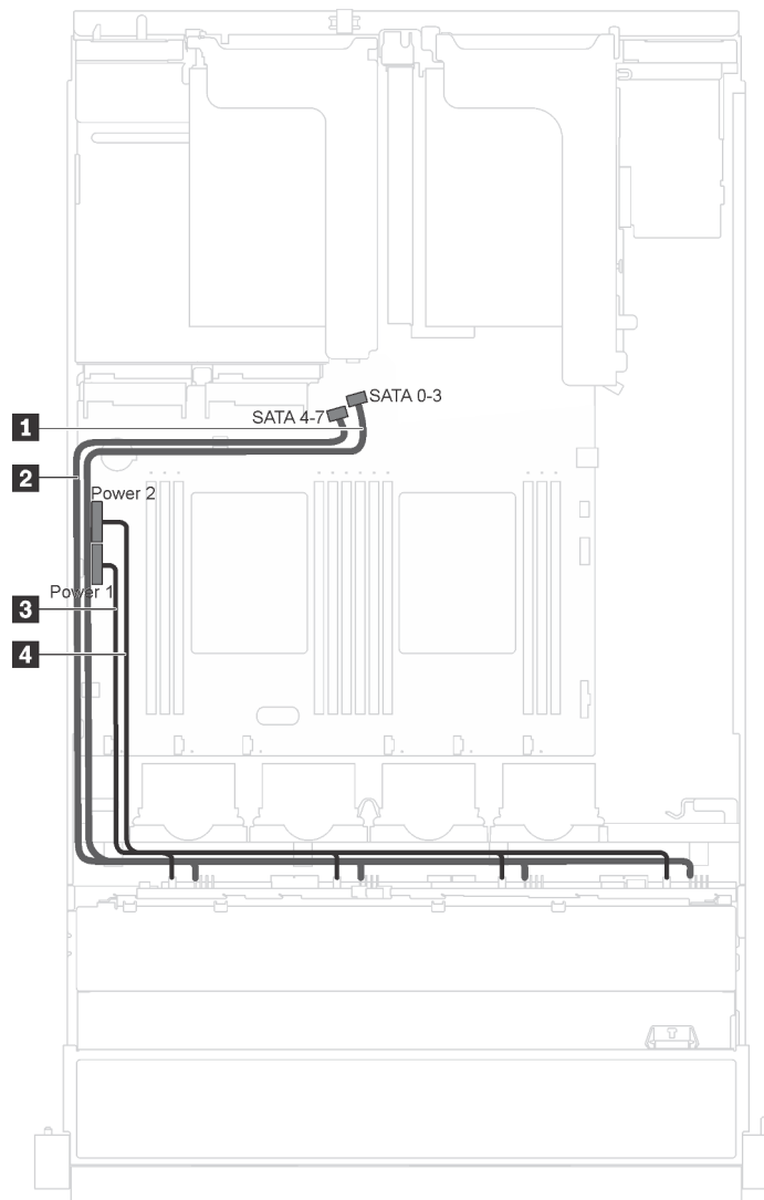
Figura 17. Roteamento de cabos para modelos de servidor com oito unidades simple-swap de 3,5 polegadas
