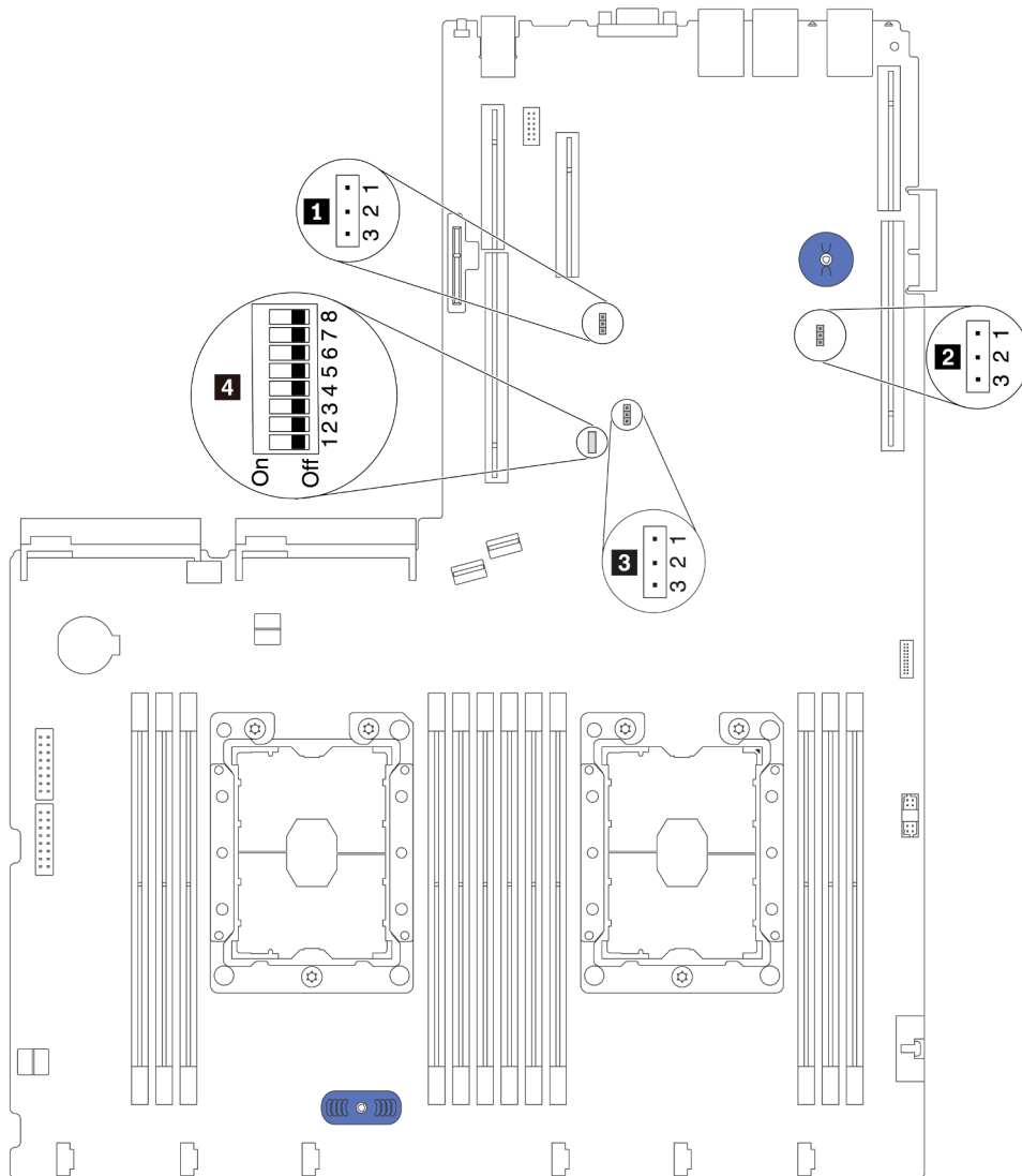
Figura 14. Comutadores e jumpers da placa-mãe
