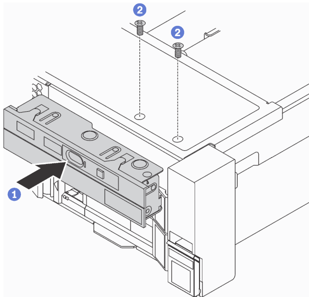
Figura 68. Instalação do conjunto de E/S frontal
