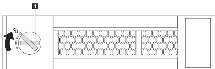
Figura 56. Abrindo a alça de uma unidade simple-swap de 3,5 polegadas
