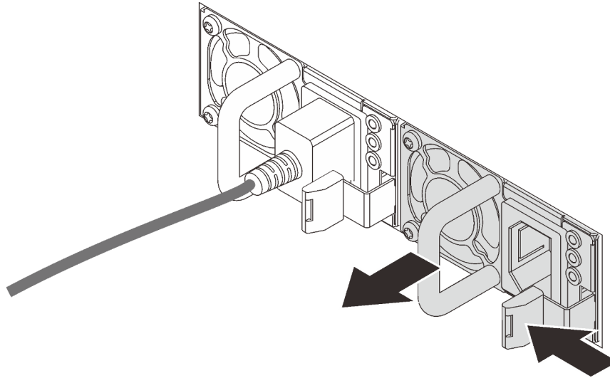
Figura 72. Remoção da fonte de alimentação hot-swap
