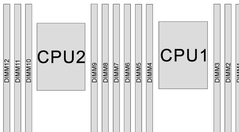
Figura 100. Slots do módulo de memória na placa-mãe
