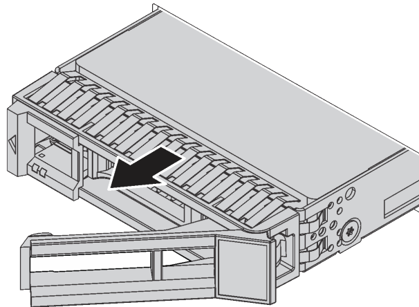
Figura 50. Remoção de uma unidade hot-swap de 2,5 polegadas
