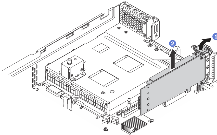
Figura 89. Removendo o adaptador PCIe da placa-mãe
