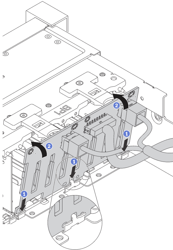
Figura 63. Instalação do backplane da unidade de 2,5 polegadas
