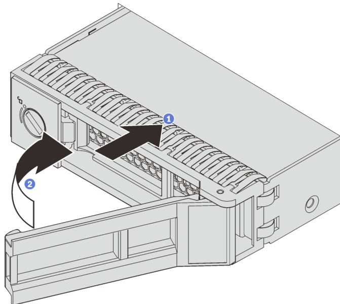
Figura 59. Instalação de unidades simple-swap
