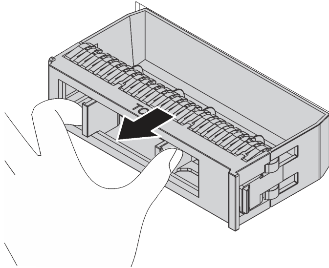
Figura 53. Remoção do preenchimento de unidade da 3,5 polegadas
