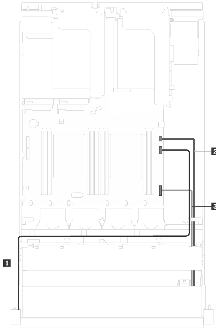
Figura 69. Conexão de cabos do conjunto de E/S frontal
