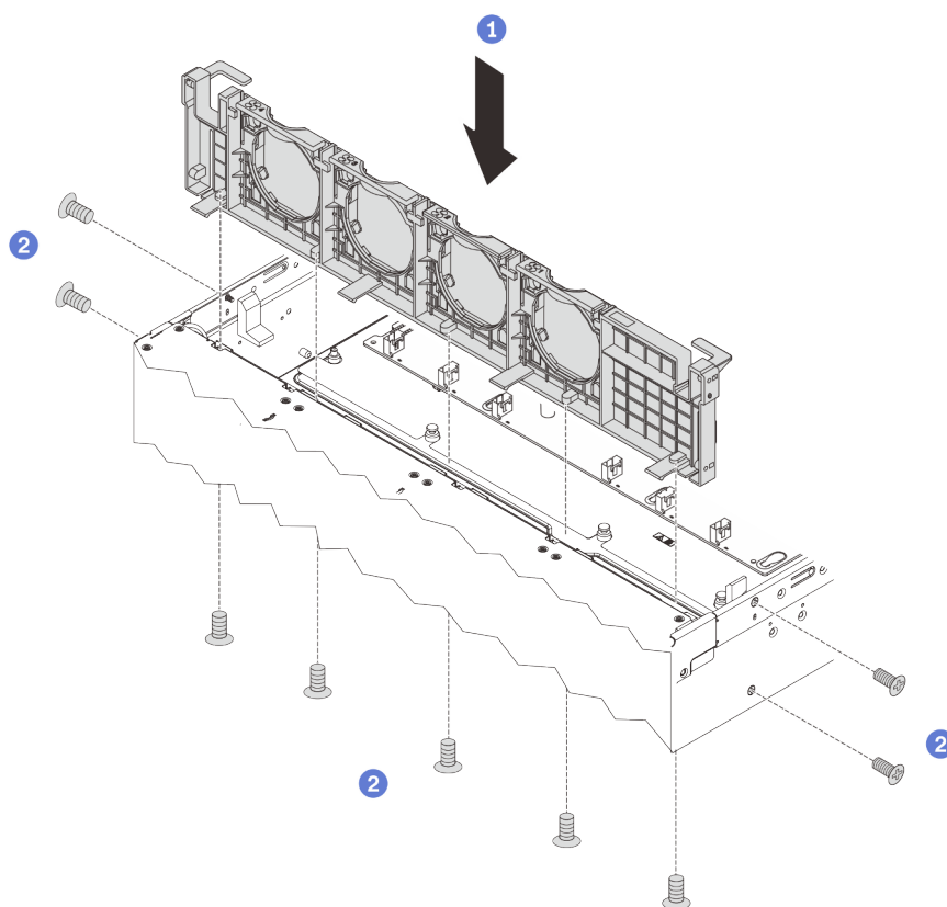
Figura 98. Instalação do compartimento do ventilador do sistema
