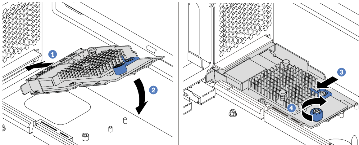
Figura 103. Instalação do adaptador LOM
