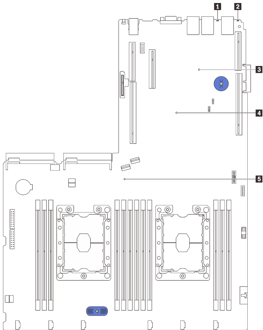
Figura 15. LEDs da placa-mãe
