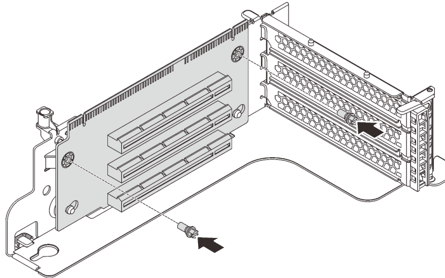
Figura 84. Instalando os dois parafusos para fixar a placa riser
