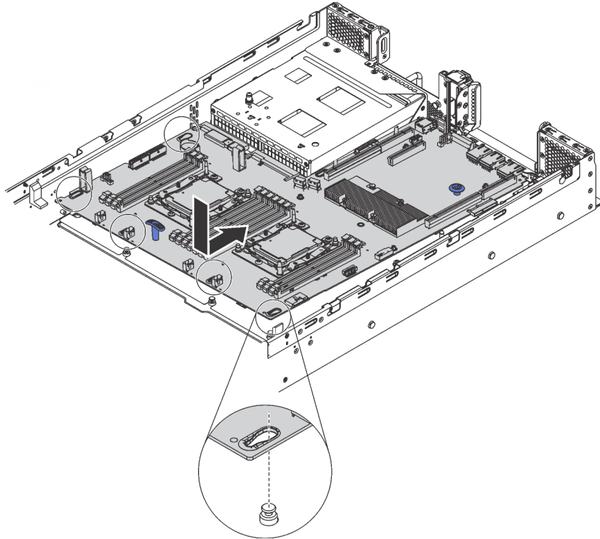
Figura 124. Instalação da placa-mãe
