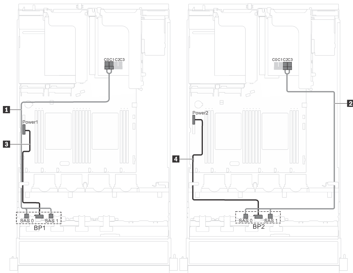
Figura 27. Roteamento de cabos para modelos de servidor com dezesseis unidades hot-swap de 2,5 polegadas, adaptador 16i e módulo de porta serial
