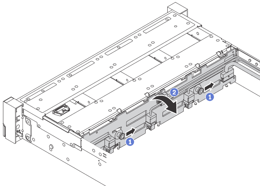
Figura 60. Remoção do painel traseiro da unidade de 3,5 polegadas
