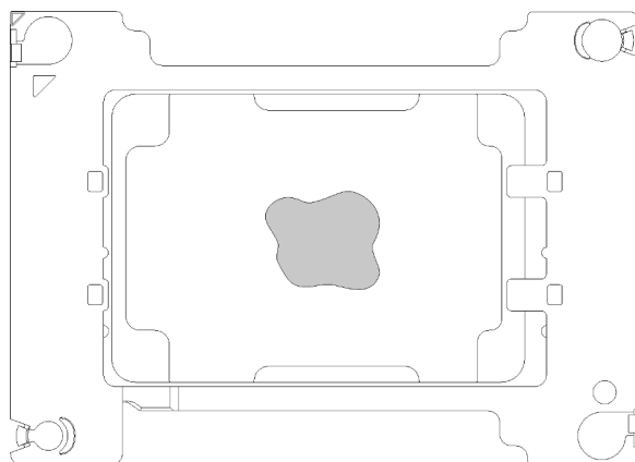
Figura 118. Formato adequado da graxa térmica
