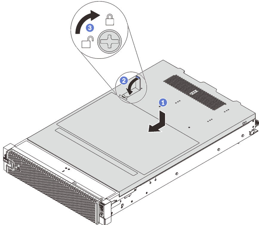
Figura 30. Instalação da tampa superior
