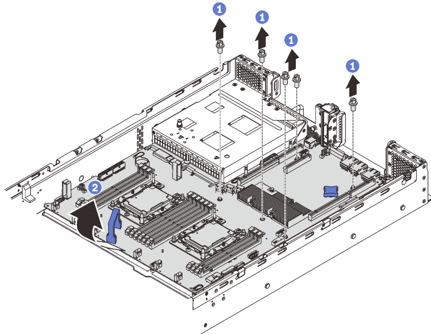
Figura 123. Remoção da placa-mãe
