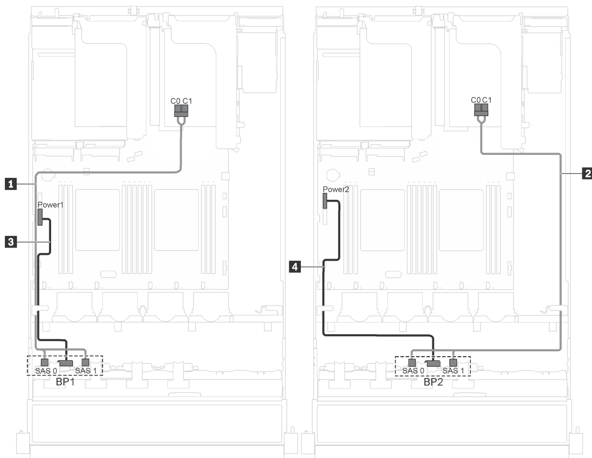
Figura 25. Roteamento de cabos para modelos de servidor com dezesseis unidades hot-swap de 2,5 polegadas, adaptadores 8i e módulo de porta serial
