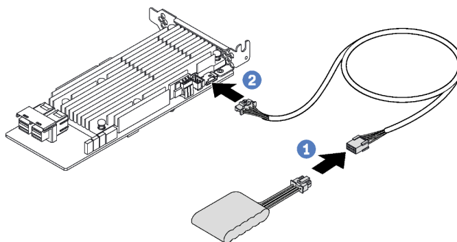
Figura 79. Conectando o módulo de supercapacitor RAID ao adaptador RAID
