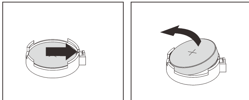
Figura 121. Remoção da bateria CMOS
