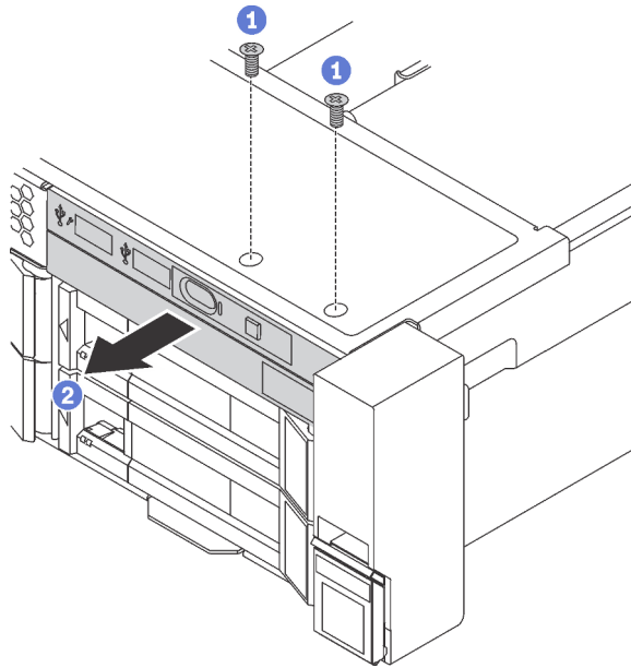
Figura 67. Remoção do conjunto de E/S frontal
