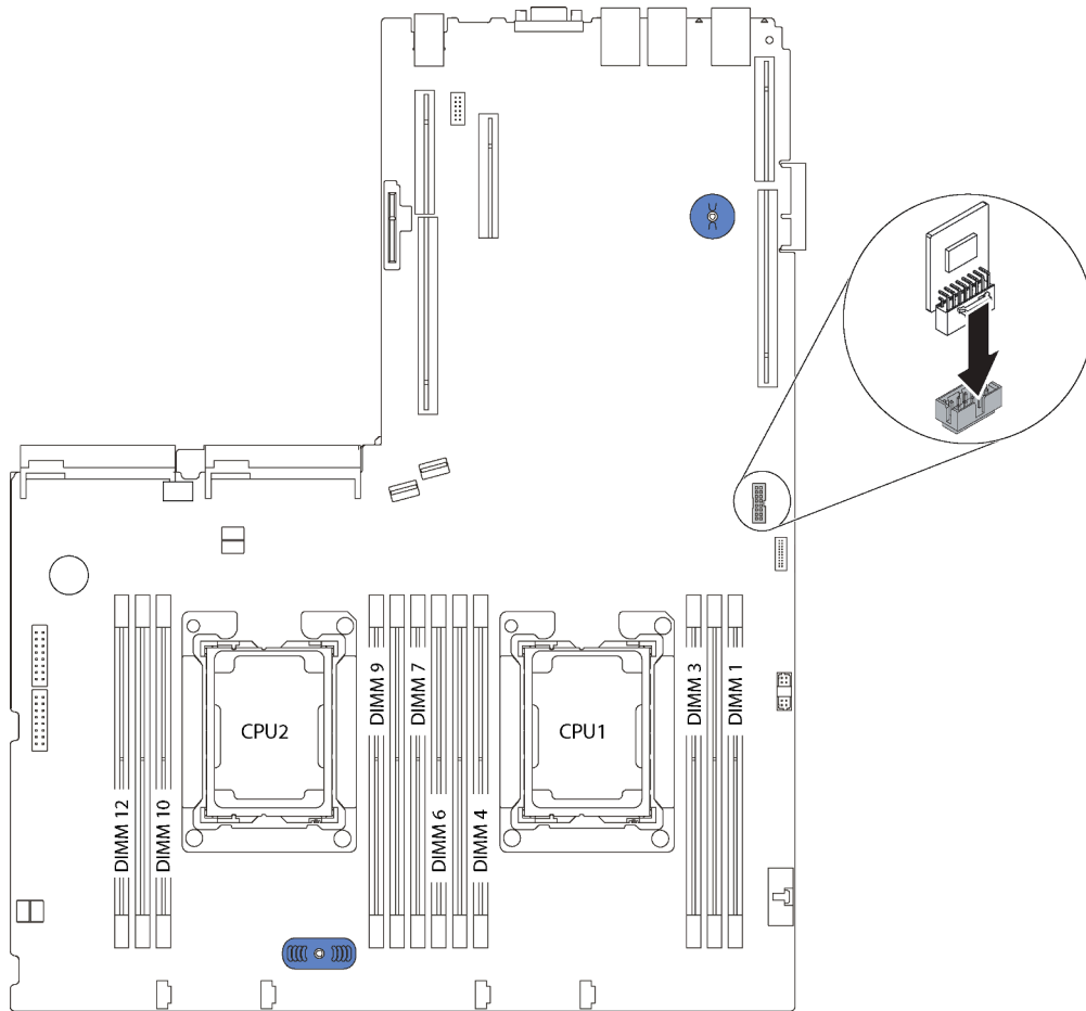
Figura 113. Instalação do adaptador TCM/TPM
