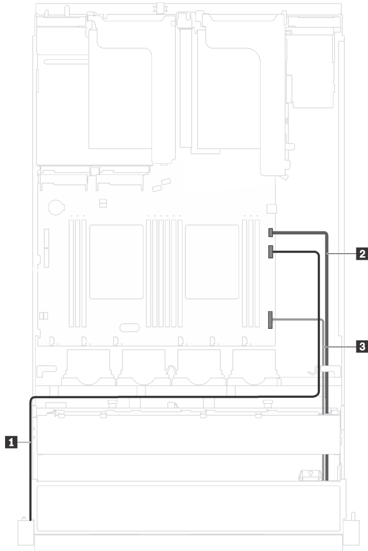
Figura 39. Conexão de cabos do conector VGA, dos conectores USB frontais e do painel de informações do operador nas travas do rack
