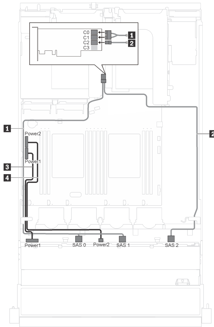
Figura 20. Roteamento de cabos para modelos de servidor com doze unidades hot-swap de 3,5 polegadas e adaptador 16i
