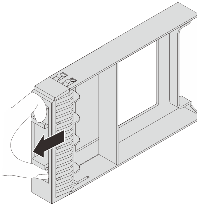
Figura 52. Remoção do preenchimento da unidade de 2,5 polegadas
