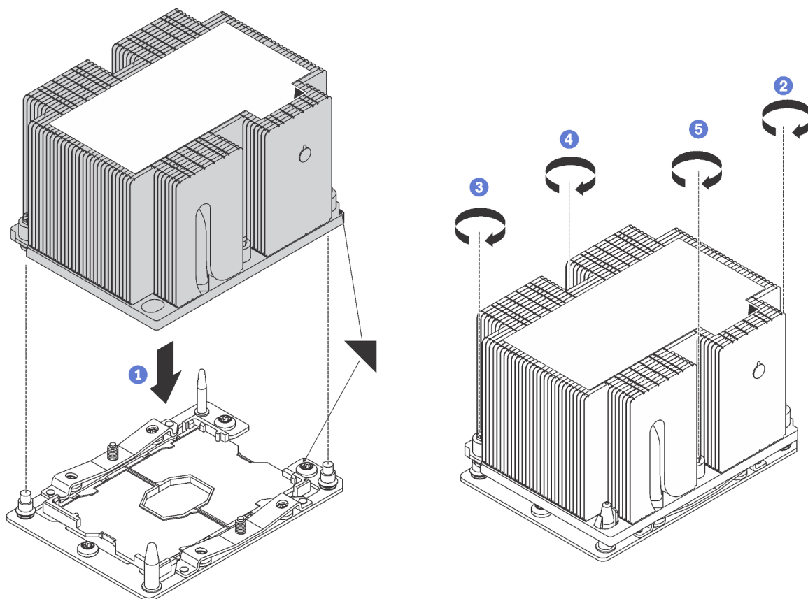
Figura 120. Instalando um PHM
