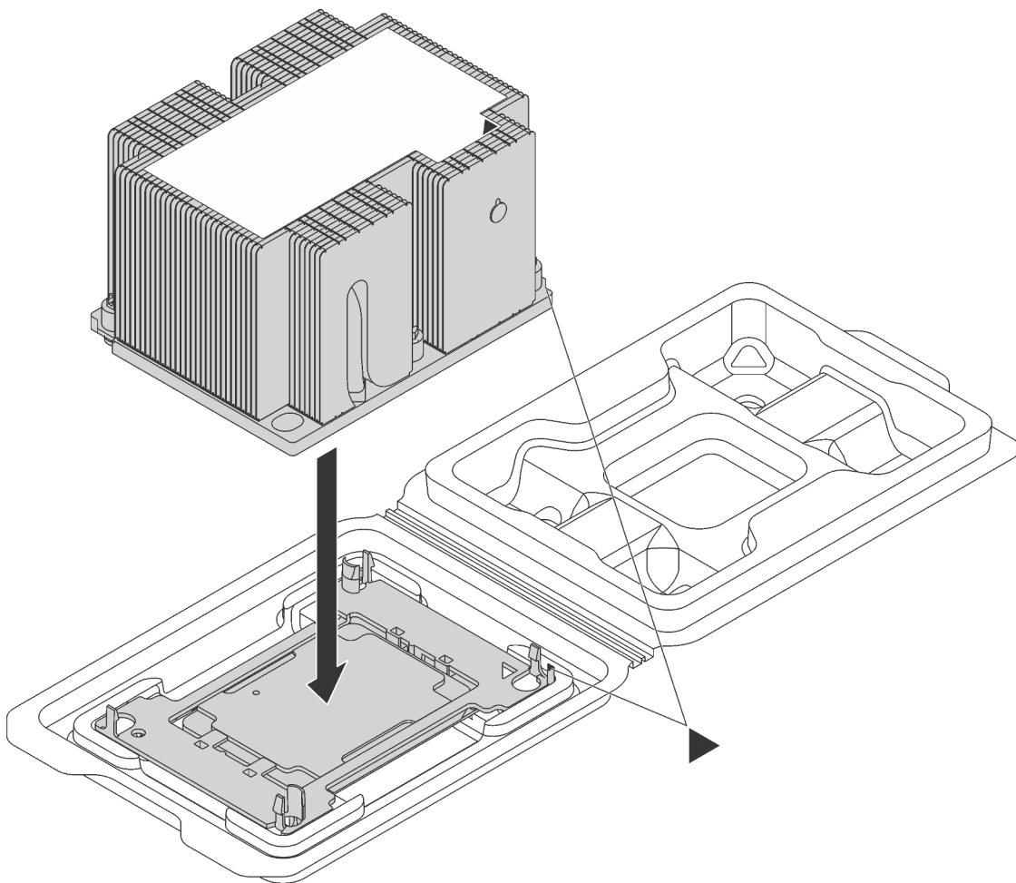
Figura 119. Montando um PHM na bandeja de remessa
