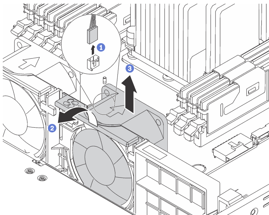
Figura 95. Remoção do ventilador do sistema
