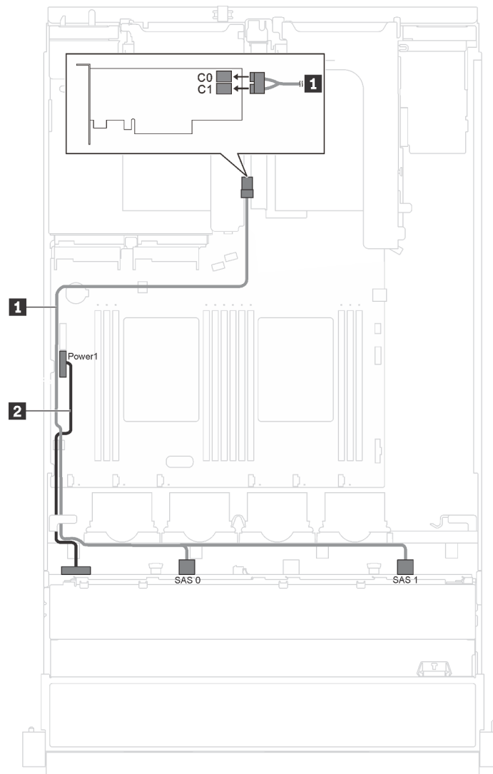
Figura 18. Roteamento de cabos para modelos de servidor com oito unidades hot-swap de 3,5 polegadas
