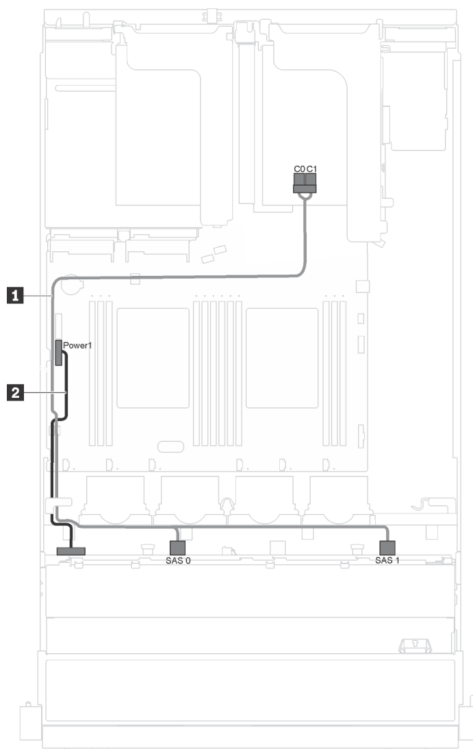
Figura 19. Roteamento de cabos para modelos de servidor com oito unidades hot-swap de 3,5 polegadas e módulo de porta serial
