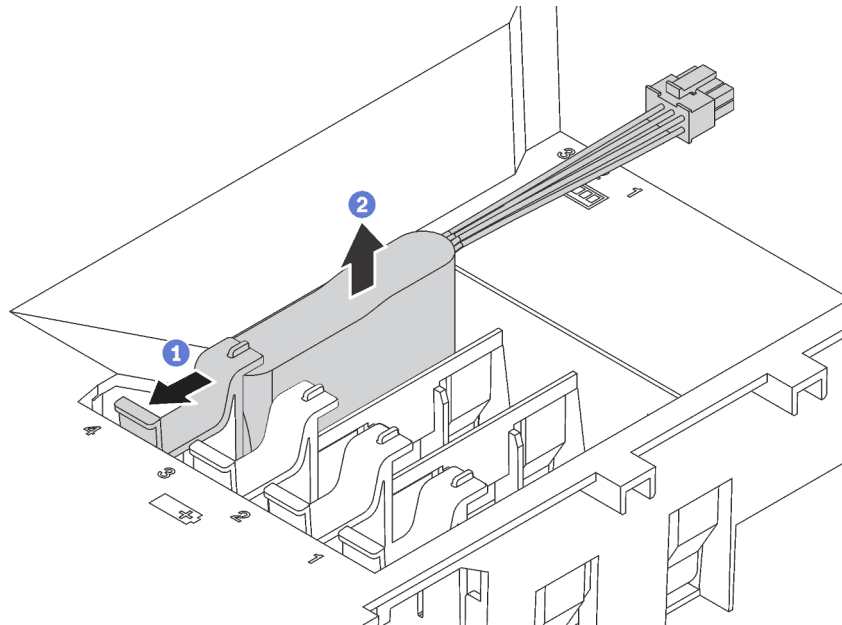
Figura 77. Remoção do módulo de supercapacitor RAID
