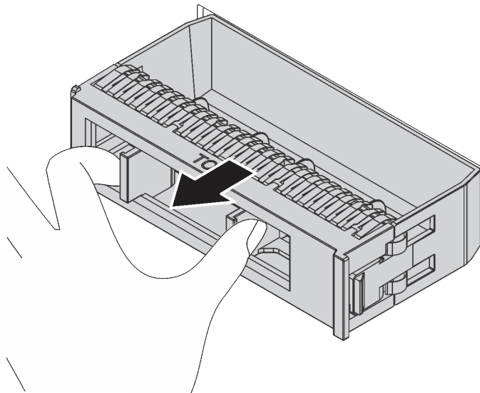
Figura 58. Remoção do preenchimento de unidade
