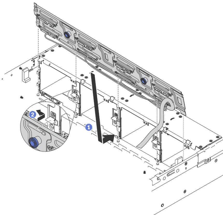
Figura 65. Instalação do conjunto de placa traseira de unidade simple-swap de 3,5 polegadas
