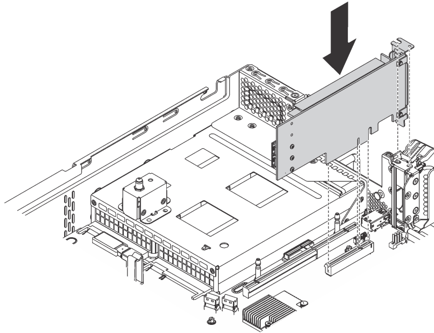
Figura 90. Instalando um adaptador PCIe na placa-mãe
