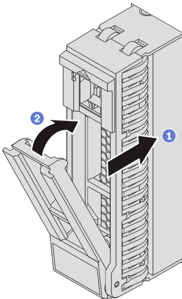
Figura 54. Instalação de uma unidade hot-swap de 2,5 polegadas
