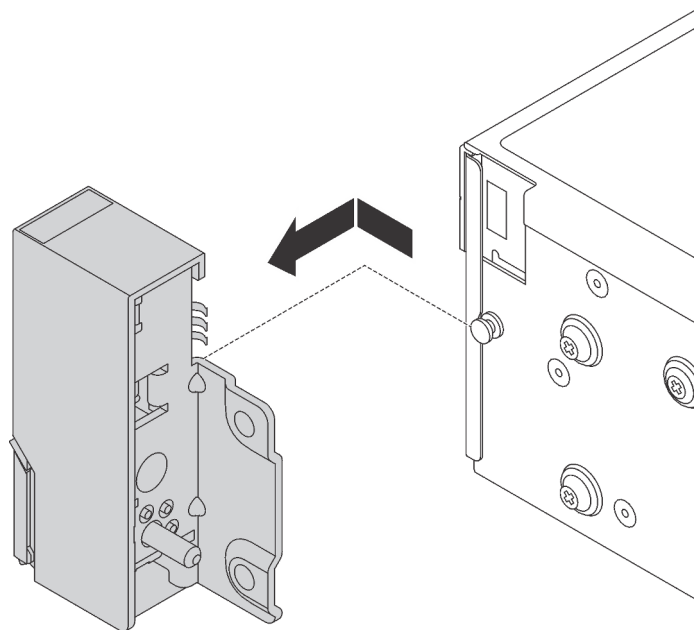
Figura 42. Remoção da trava do rack
