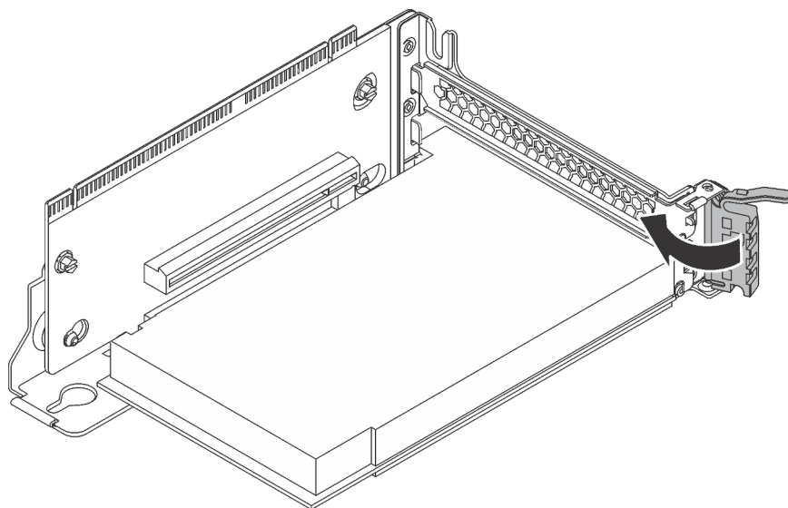
Figura 92. Girando a trava de retenção para a posição fechada
