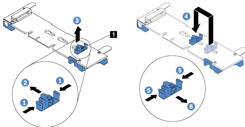
Figura 111. Ajuste do retentor M.2
