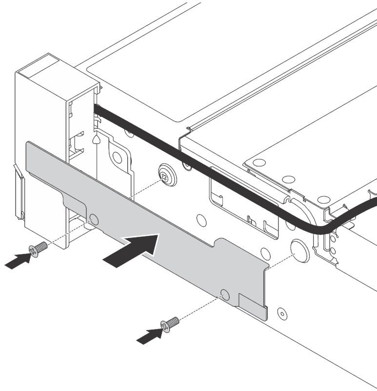
Figura 45. Instalação do retentor de cabos
