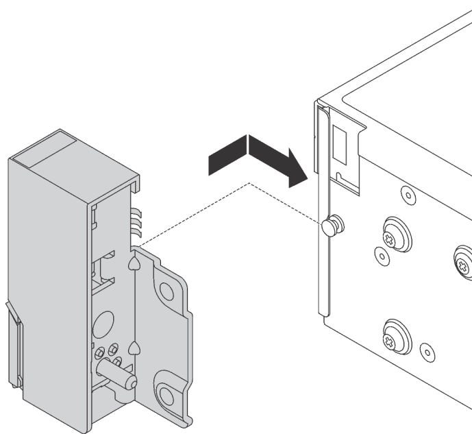
Figura 43. Instalação da trava do rack
