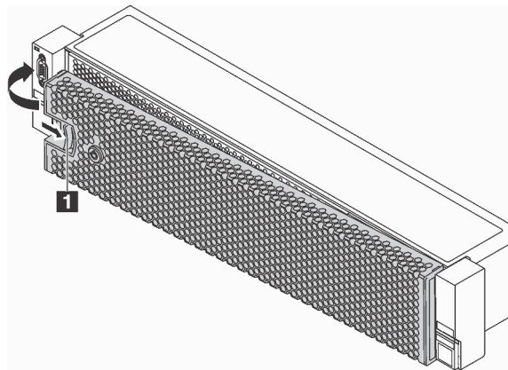
Figura 36. Instalação do painel de segurança
