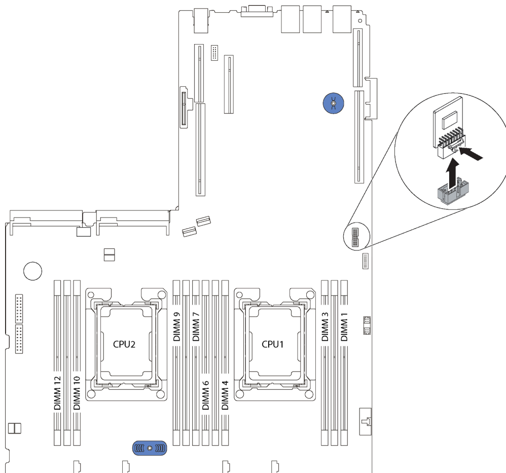
Figura 112. Remoção do adaptador TCM/TPM
