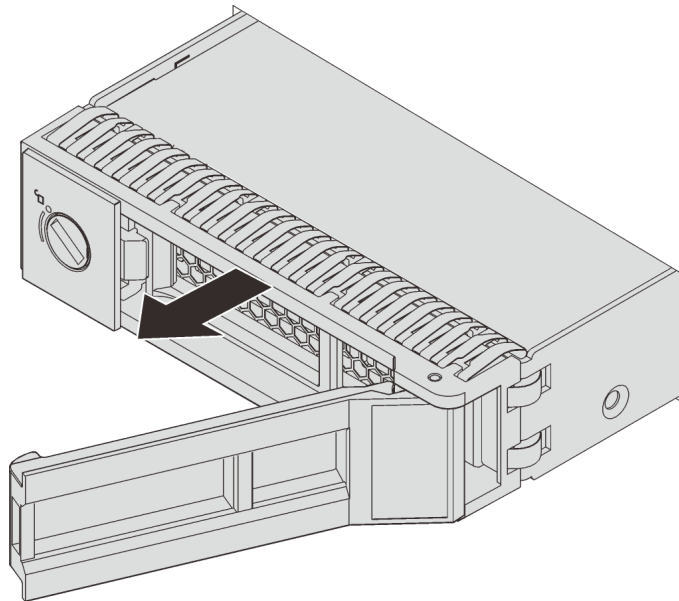
Figura 57. Remoção de uma unidade simple-swap de 3,5 polegadas
