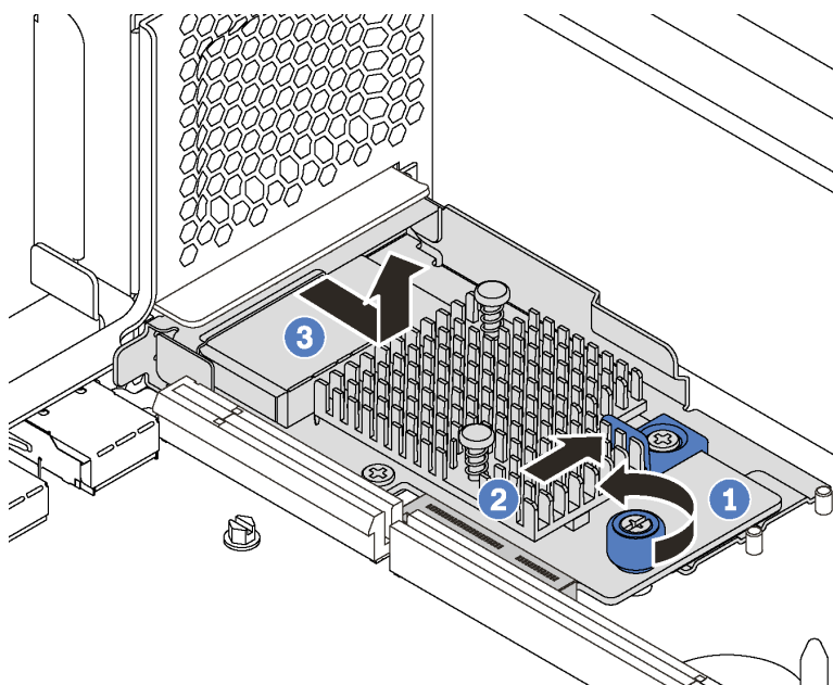
Figura 102. Remoção do adaptador LOM
