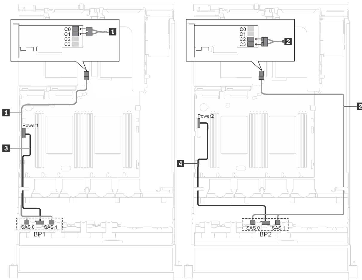
Figura 26. Roteamento de cabos para modelos de servidor com dezesseis unidades hot-swap de 2,5 polegadas e adaptador 16i
