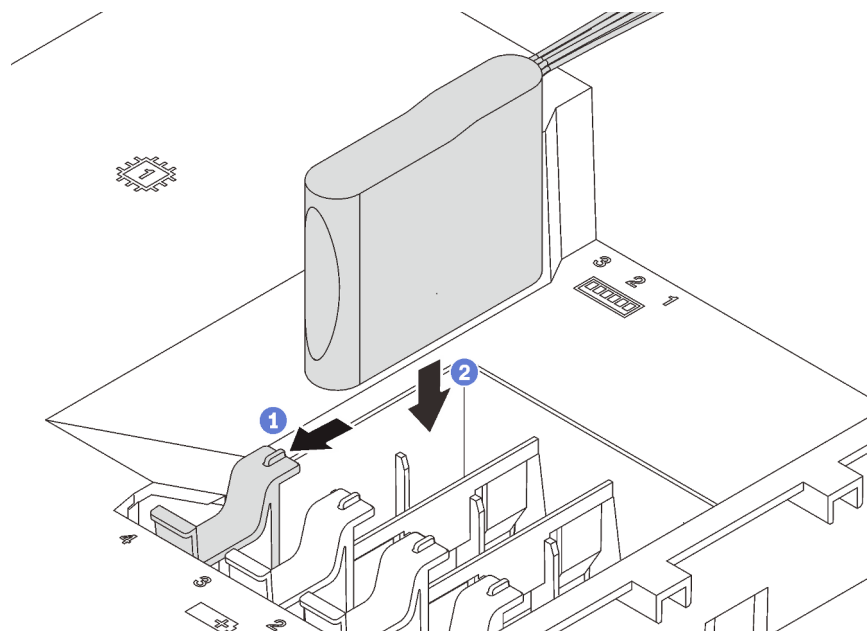
Figura 78. Instalação do módulo de supercapacitor RAID
