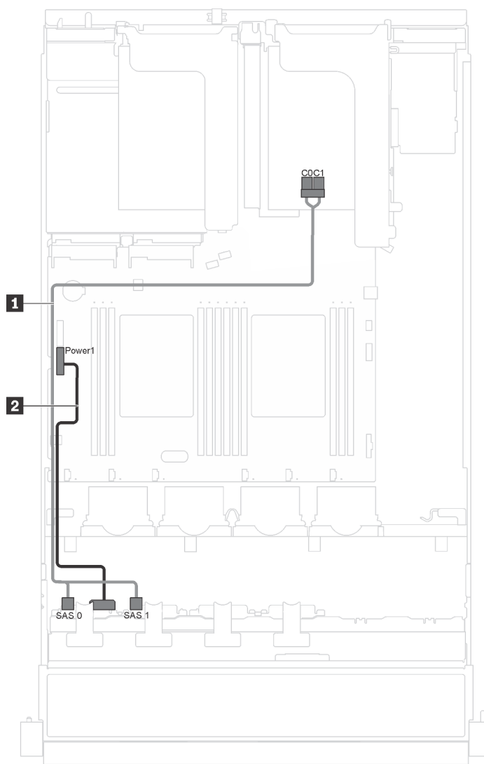
Figura 23. Roteamento de cabos para modelos de servidor com oito unidades hot-swap de 2,5 polegadas e módulo de porta serial
