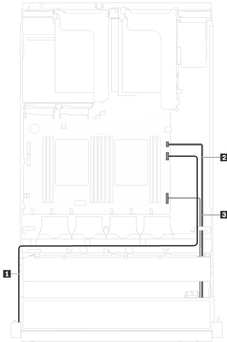
Figura 46. Conexão de cabos do conector VGA e do conjunto de E/S frontal nas travas do rack
