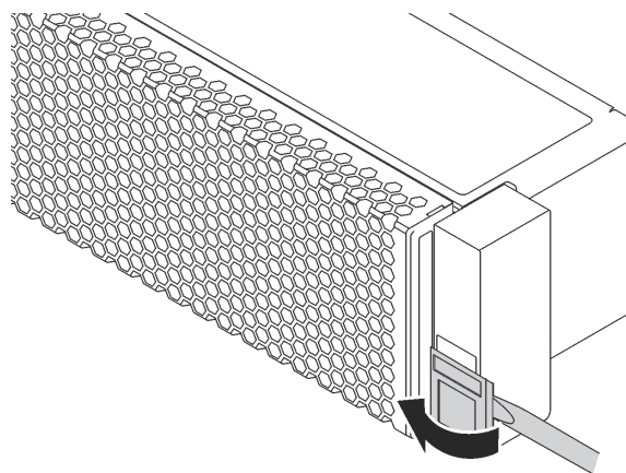
Figura 38. Remoção da placa com etiqueta de identificação
