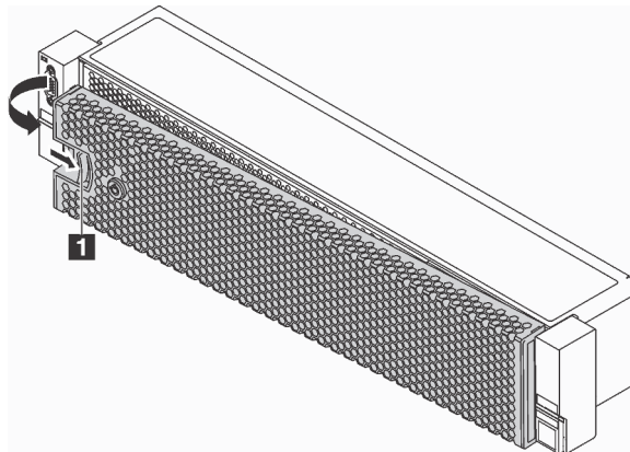
Figura 34. Remoção do painel de segurança
