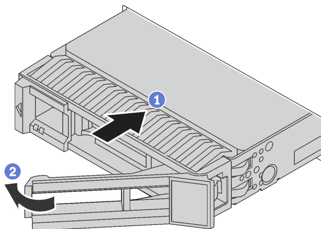
Figura 55. Instalação de uma unidade hot-swap de 3,5 polegadas
