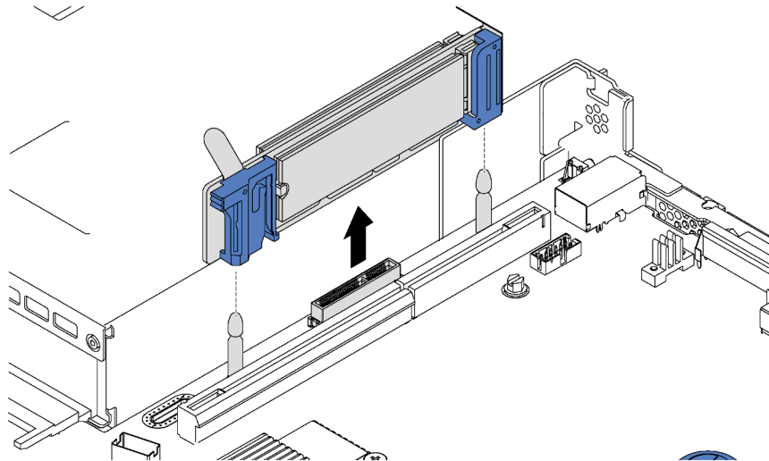
Figura 105. Remoção do painel traseiro M.2
