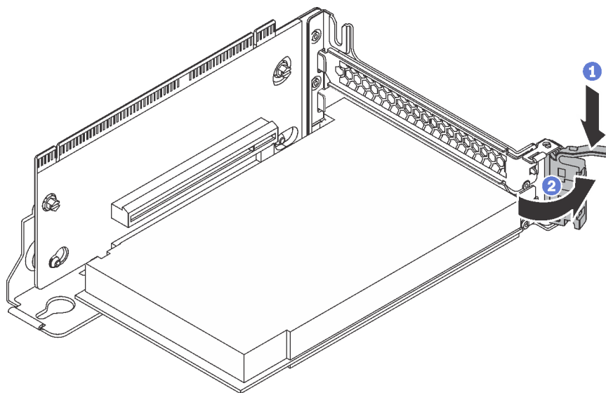
Figura 87. Abrindo a trava de retenção do adaptador PCIe
