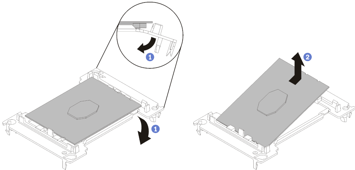
Figura 116. Removendo um retentor de processador
