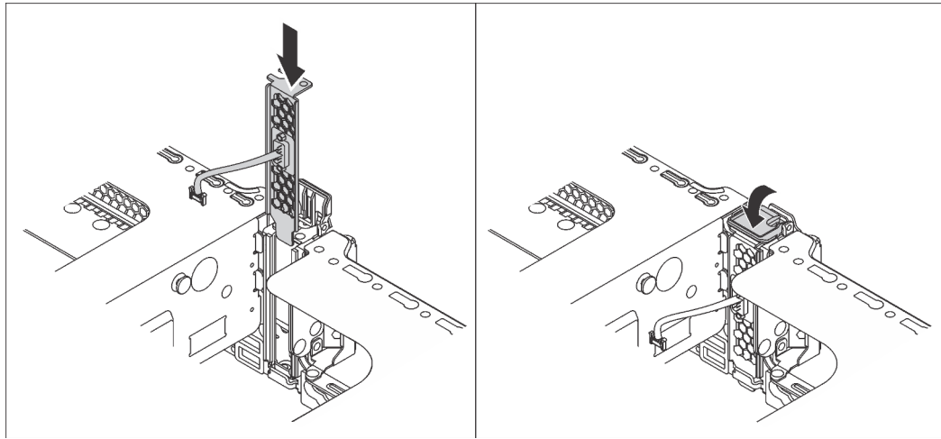
Figura 94. Instalação do módulo de porta serial
