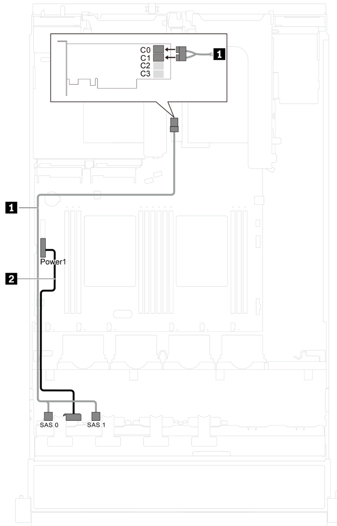
Figura 22. Roteamento de cabos para modelos de servidor com oito unidades hot-swap de 2,5 polegadas
