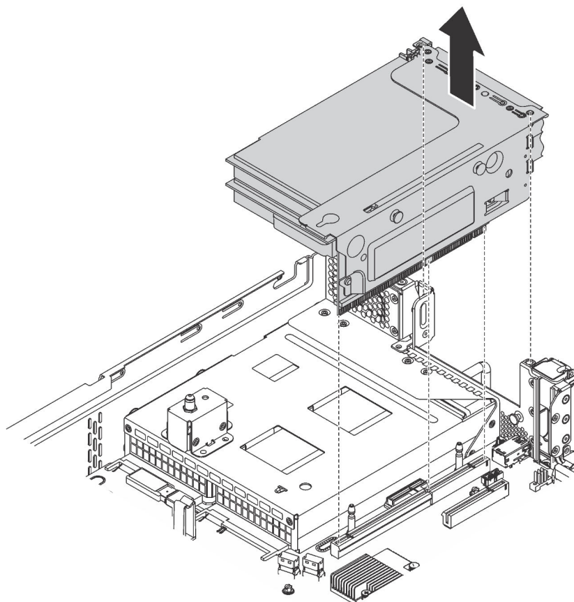
Figura 81. Remoção do conjunto da placa riser 2
