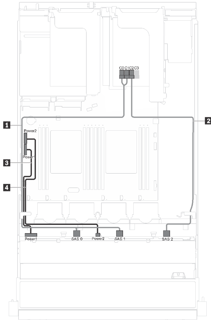
图 19. 配备十二个 3.5 英寸热插拔硬盘、16i 适配器和串口模块的服务器型号的线缆布放
