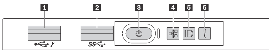
图 9. 配备 2.5 英寸硬盘插槽或八个 3.5 英寸硬盘插槽的服务器型号的正面 I/O 组合件
