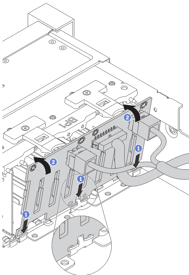
图 34. 安装 2.5 英寸硬盘背板
