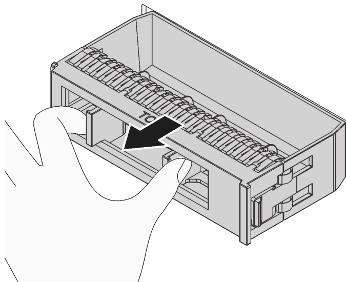
图 57. 卸下 3.5 英寸硬盘填充件
