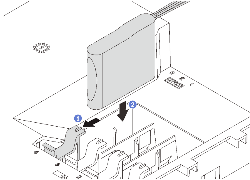
图 53. 安装 RAID 超级电容器模块
