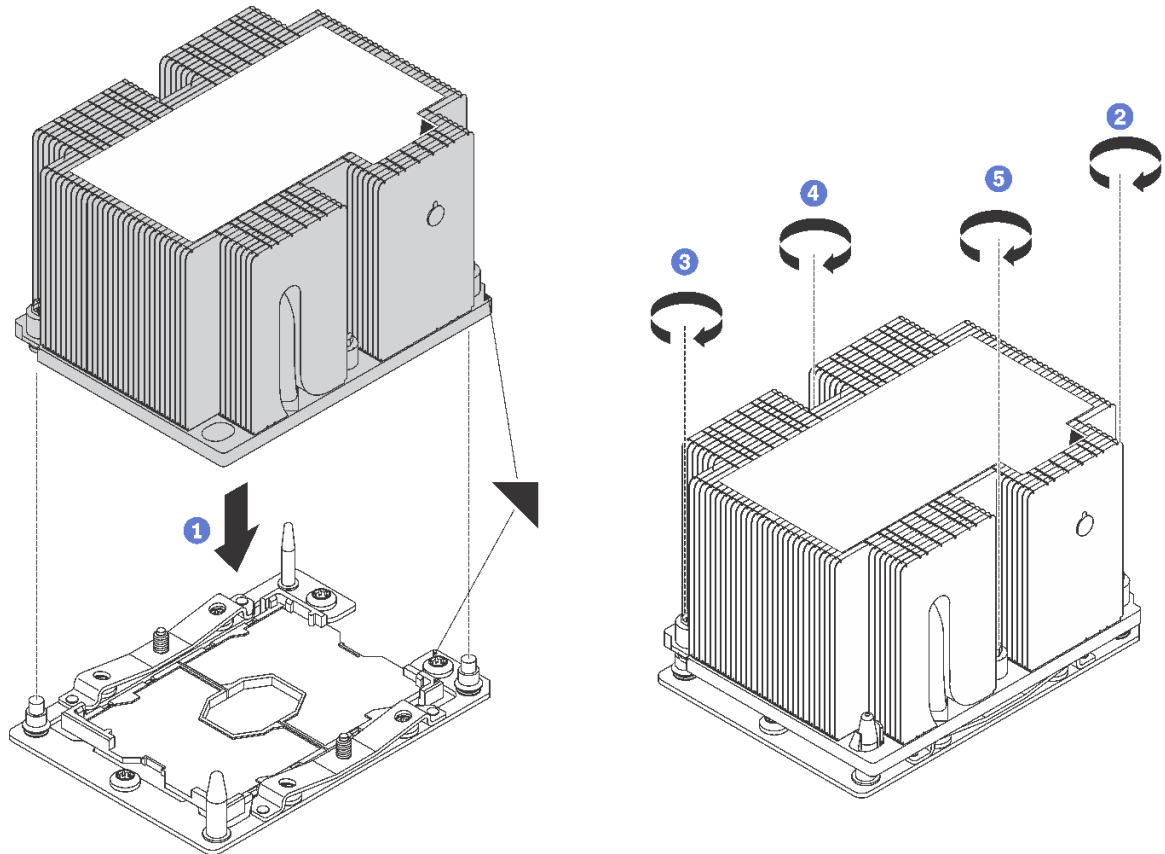
图 31. 安装 PHM
