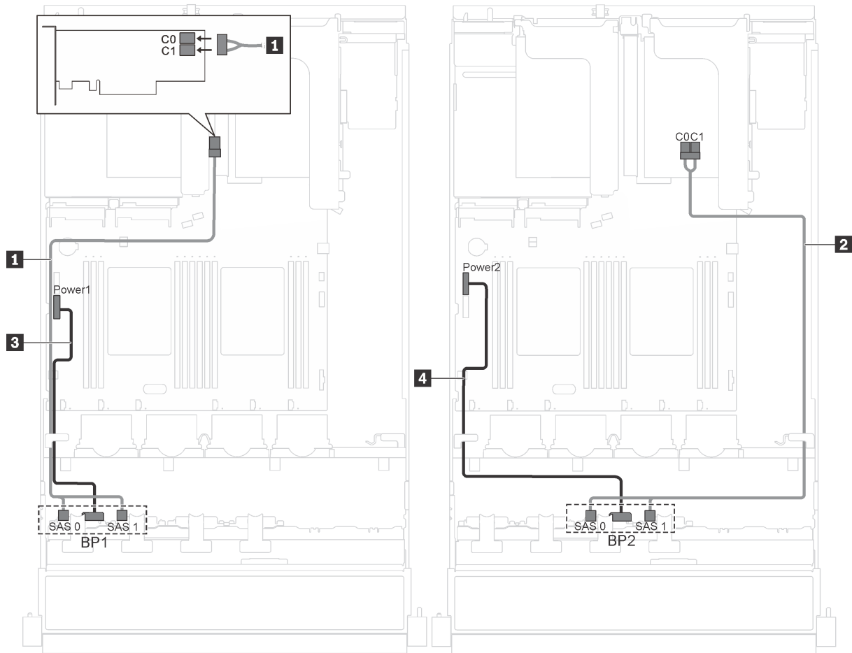
图 22. 配备十六个 2.5 英寸热插拔硬盘和两个 8i 适配器的服务器型号的线缆布放
