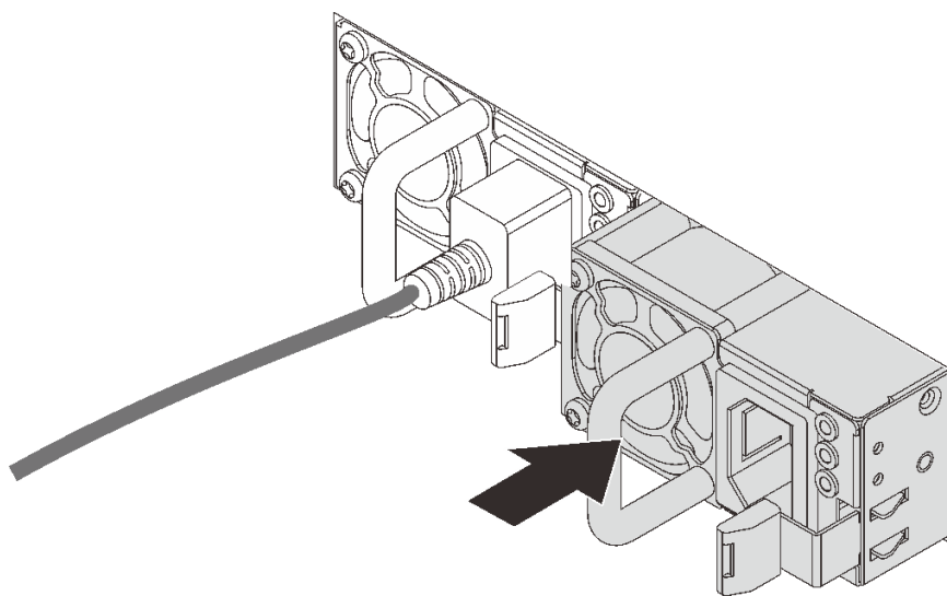
图 51. 安装热插拔电源模块
