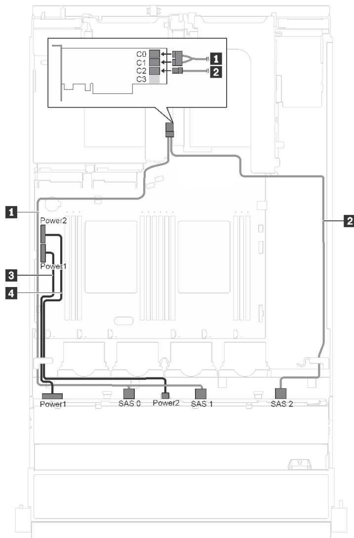
图 18. 配备十二个 3.5 英寸热插拔硬盘和 16i 适配器的服务器型号的线缆布放
