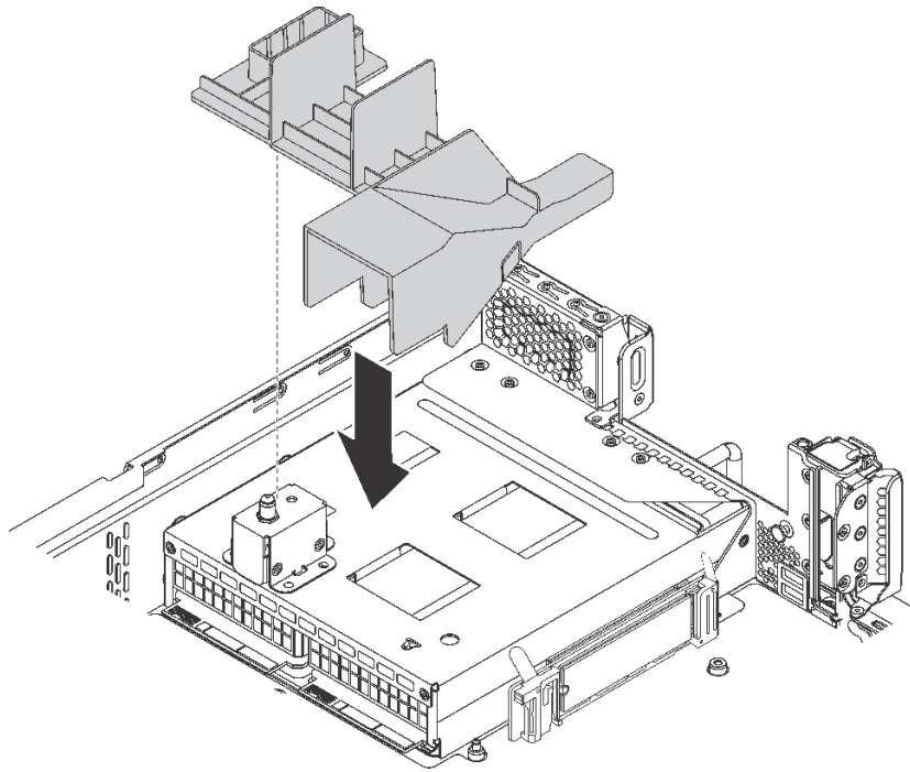
图 47. M.2 硬盘导风罩安装
