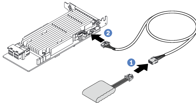
图 54. 将 RAID 超级电容器模块连接到 RAID 适配器
