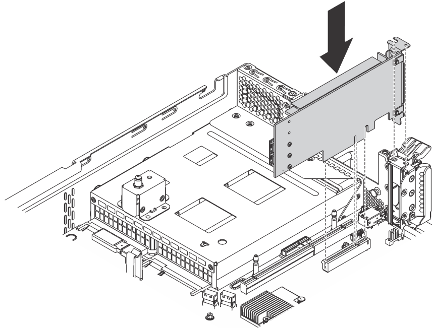
图 43. 将 PCIe 适配器安装到主板上
