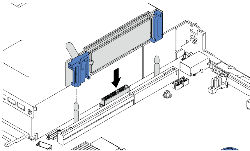
图 46. 安装 M.2 背板
