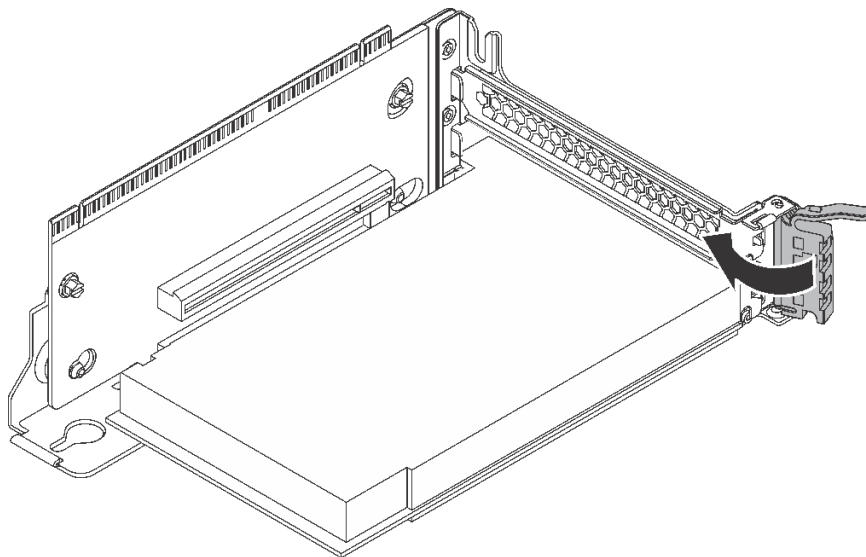
图 42. 将固定滑锁旋转至闭合位置
