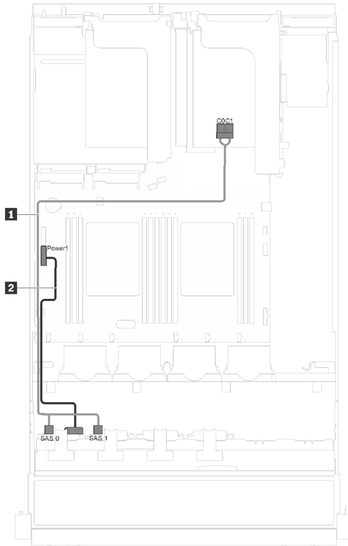
图 21. 配备八个 2.5 英寸热插拔硬盘和串口模块的服务器型号的线缆布放
