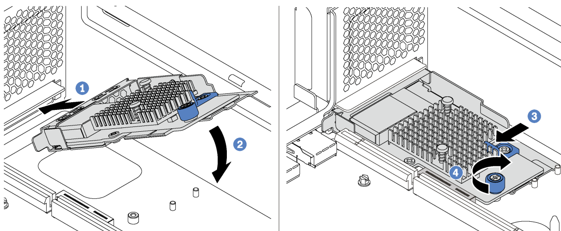
图 40. 安装 LOM 适配器
