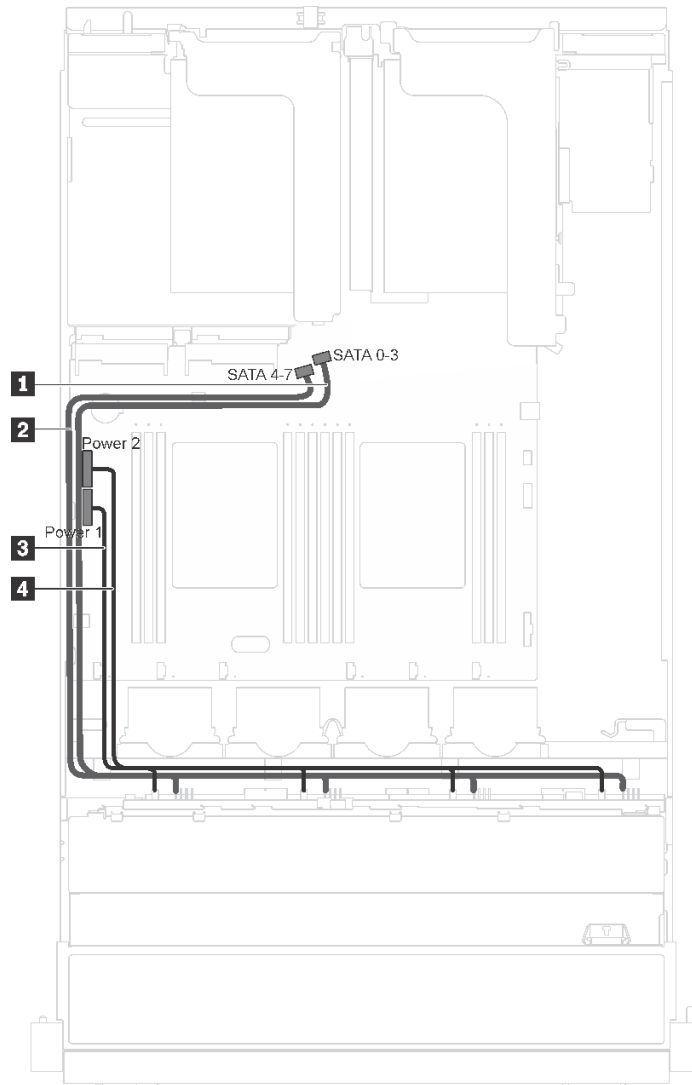
图 15. 配备八个 3.5 英寸易插拔硬盘的服务器型号的线缆布放
