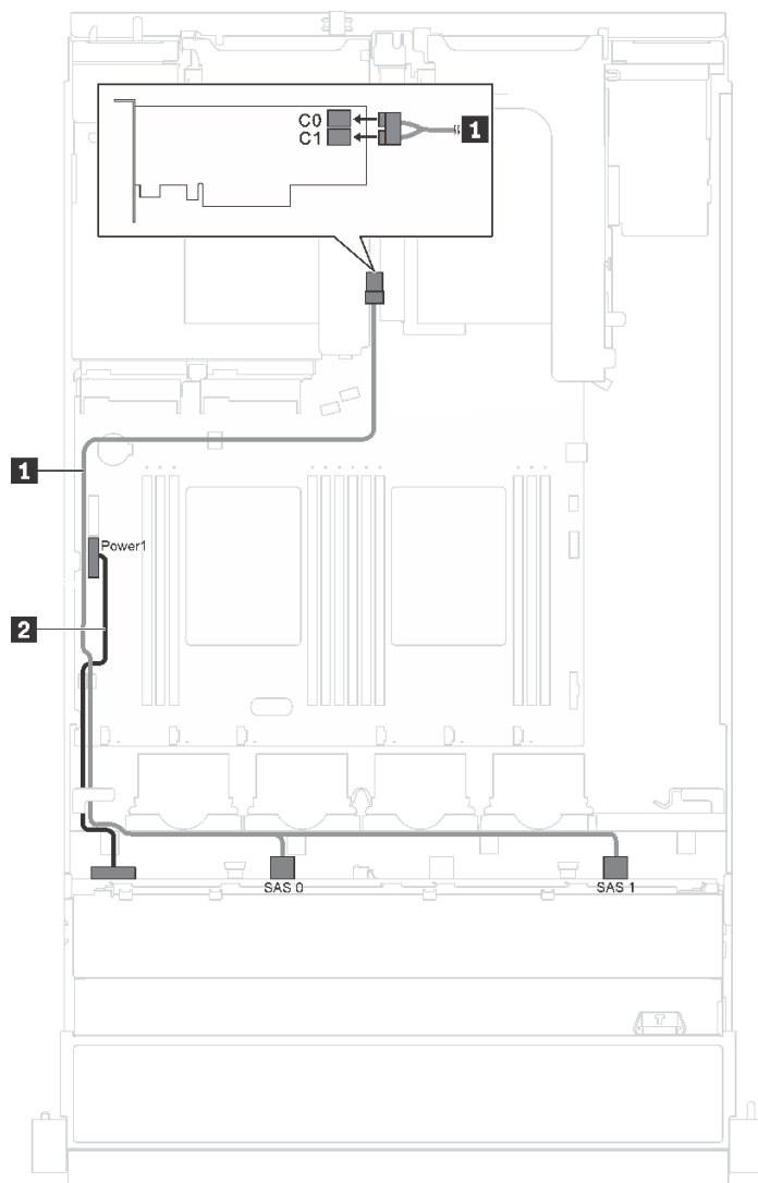
图 16. 配备八个 3.5 英寸热插拔硬盘的服务器型号的线缆布放
