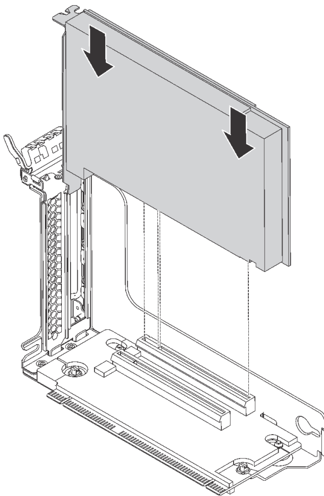
图 41. 将 PCIe 适配器安装到转接卡组件上
