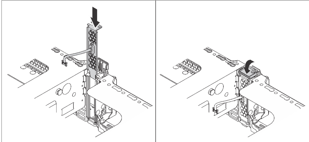
图 39. 安装串口模块
