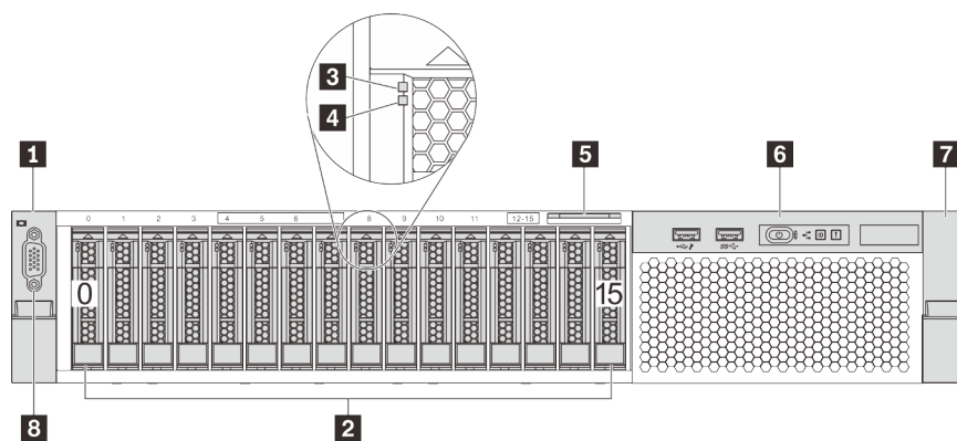
图 5. 配备十六个 2.5 英寸热插拔硬盘 (0-15) 的服务器型号的前视图
