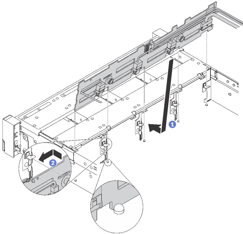
图 36. 安装 3.5 英寸硬盘背板
