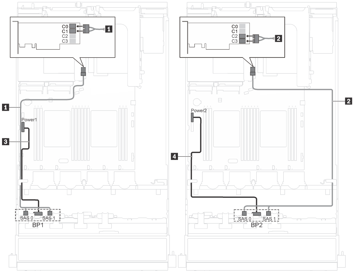
图 24. 配备十六个 2.5 英寸热插拔硬盘和 16i 适配器的服务器型号的线缆布放
