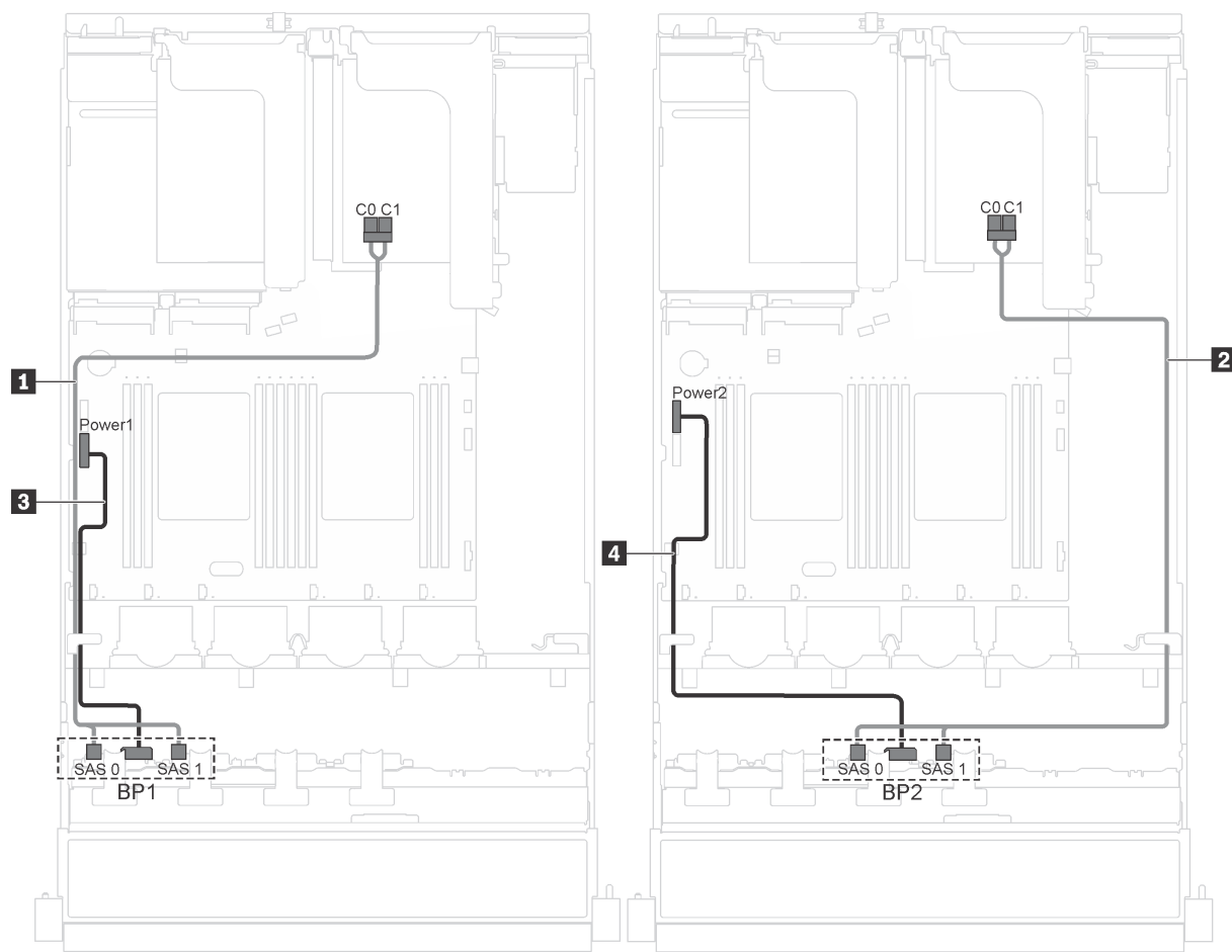
图 23. 配备十六个 2.5 英寸热插拔硬盘、8i 适配器和串口模块的服务器型号的线缆布放
