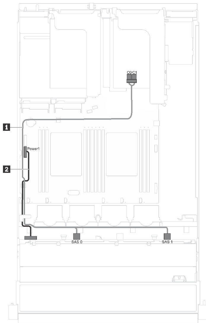
图 17. 配备八个 3.5 英寸热插拔硬盘和串口模块的服务器型号的线缆布放
