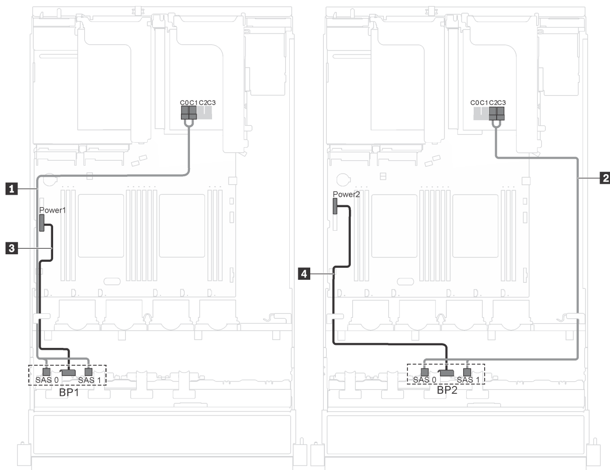
图 25. 配备十六个 2.5 英寸热插拔硬盘、16i 适配器和串口模块的服务器型号的线缆布放
