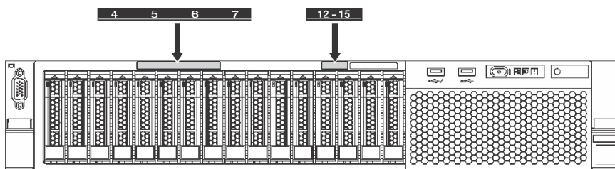
图 35. 装有两个 SATA/SAS 背板的服务器型号的硬盘插槽标签
