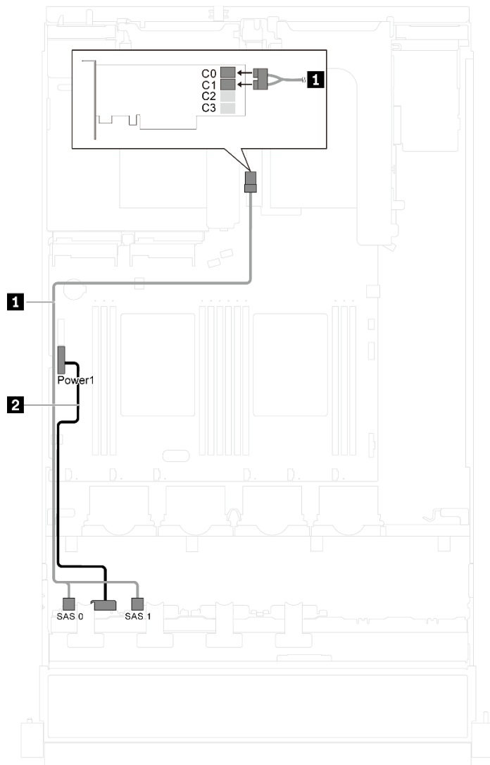
图 20. 配备八个 2.5 英寸热插拔硬盘的服务器型号的线缆布放
