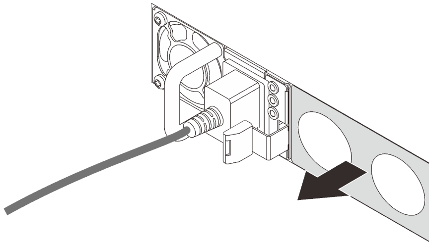
Abbildung 102. Entfernen der Abdeckblende für Hot-Swap-Netzteil
