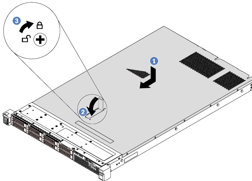
Abbildung 27. Installation der oberen Abdeckung
