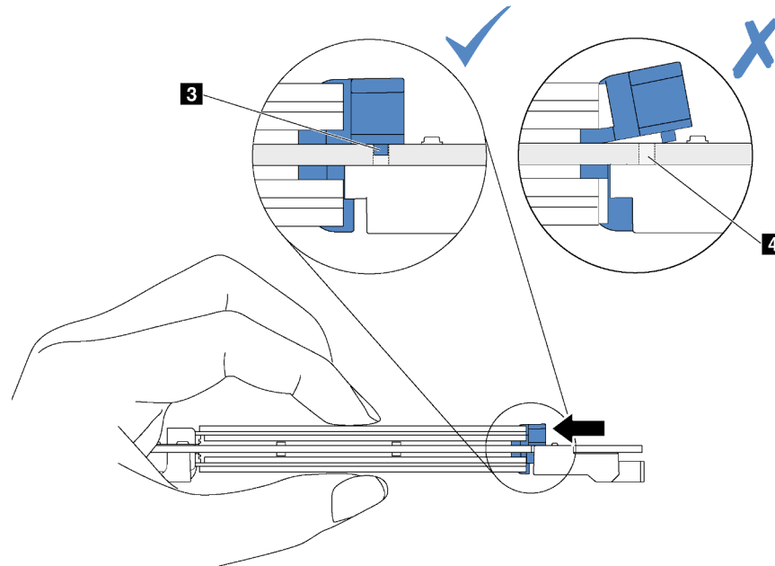
Abbildung 87. Anweisungen zum Schieben der Halterung
