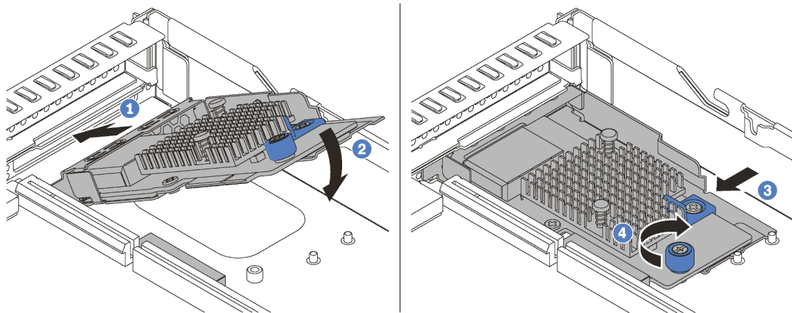
Abbildung 54. Installieren eines LOM-Adapters
