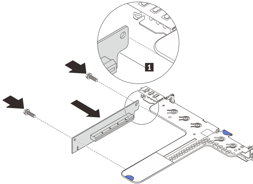
Abbildung 57. Installation einer Adapterkarte
