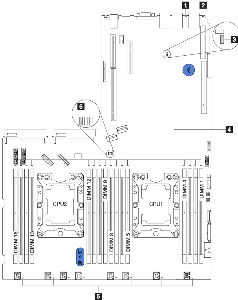
Abbildung 12. Anzeigen auf der Systemplatine
