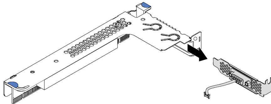
Abbildung 78. Serielles Anschlussmodul entfernen
