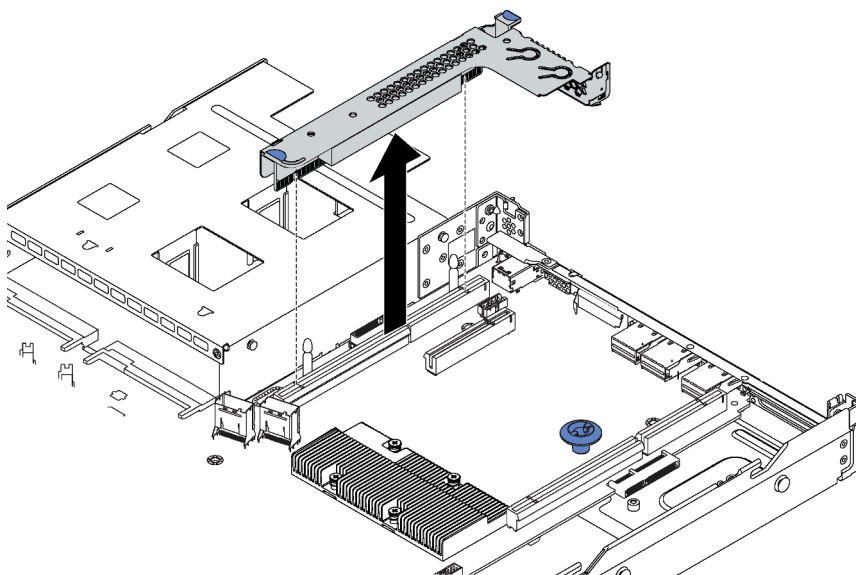
Abbildung 79. Entfernen der Adapterkartenbaugruppe
