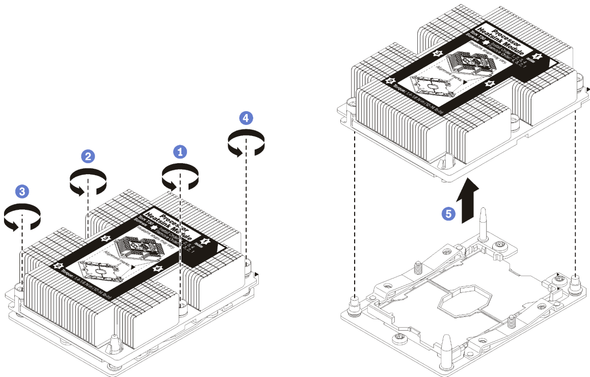
Abbildung 104. Entfernen des PHM
