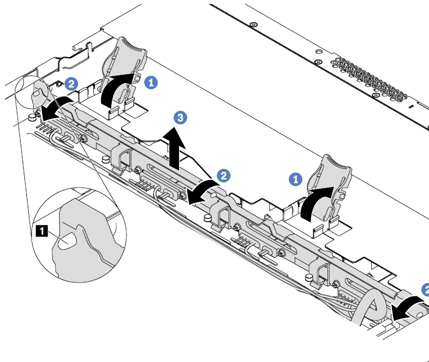
Abbildung 71. Rückwandbaugruppe für Simple-Swap-Laufwerke entfernen
