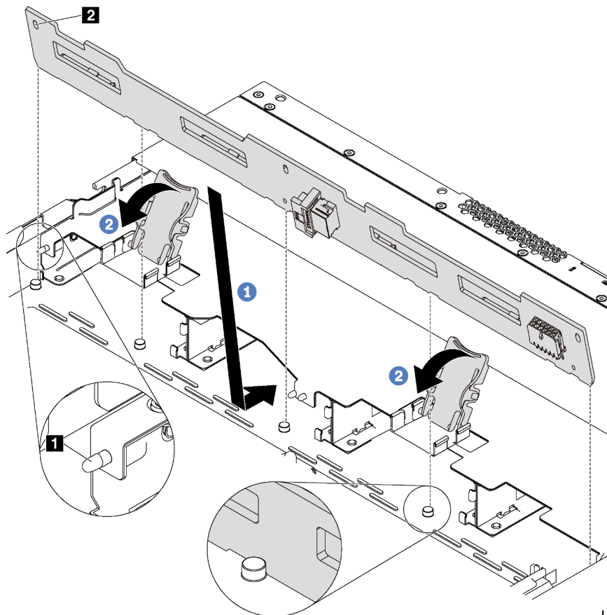
Abbildung 66. Installation einer Rückwandplatine für vier 3,5-Zoll-Hot-Swap-Laufwerke
