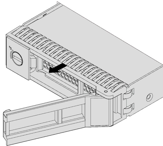
Abbildung 51. Entfernung eines Simple-Swap-Laufwerks
