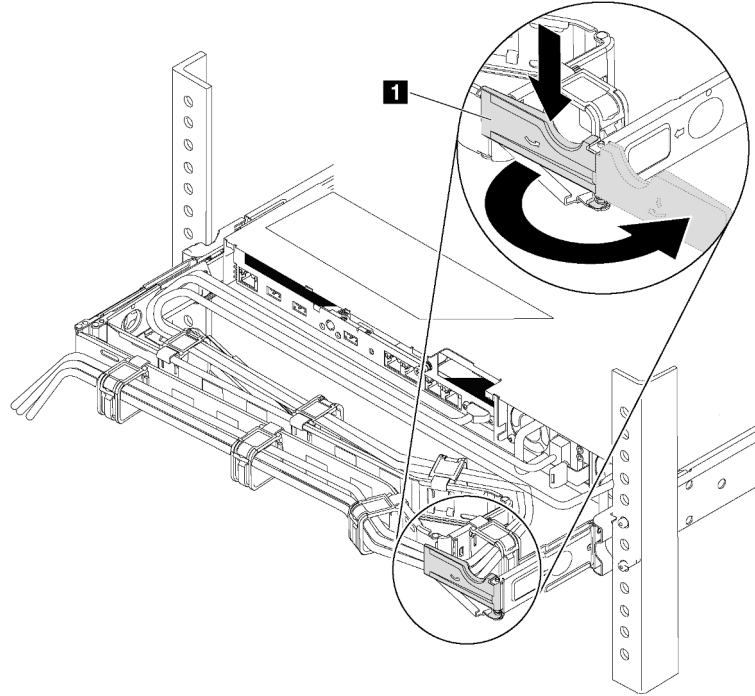
Abbildung 101. CMA-Anpassung
