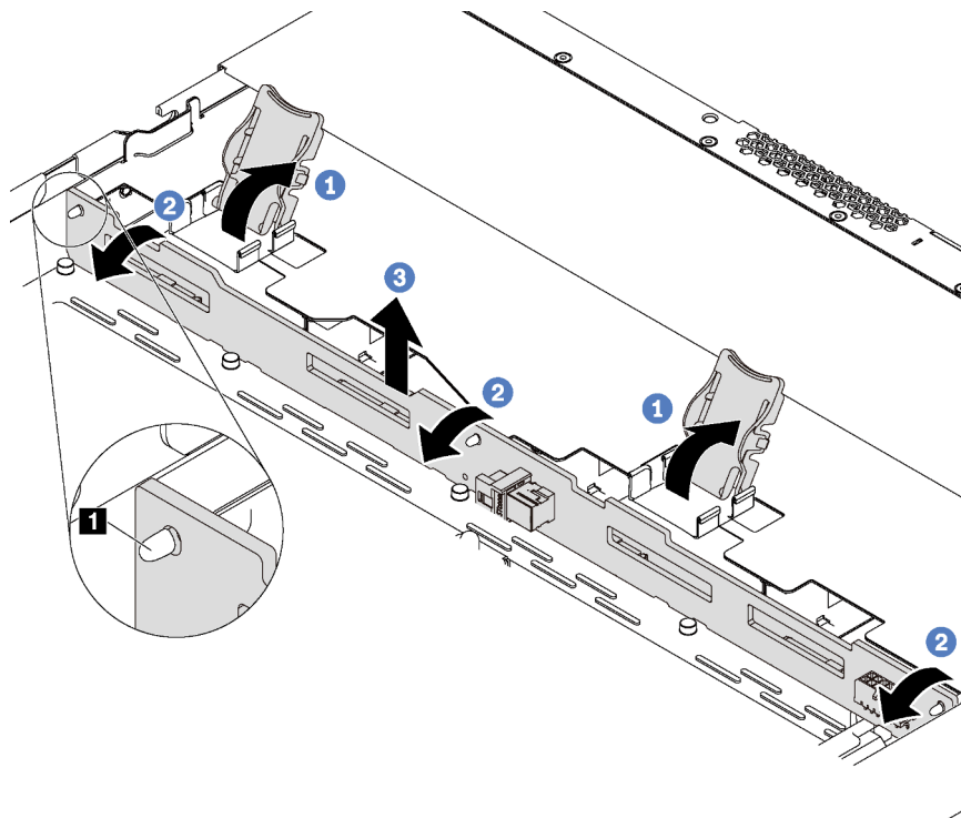
Abbildung 65. Entfernen der Rückwandplatte für vier 3,5-Zoll-Hot-Swap-Laufwerke
