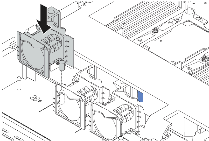
Abbildung 42. Installation des Systemlüfters
