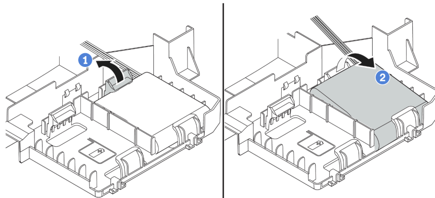
Abbildung 89. Entfernen des RAID-Superkondensatormoduls
