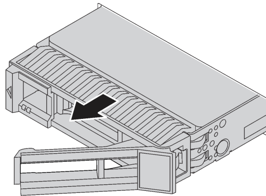
Abbildung 47. Entfernen eines Hot-Swap-Laufwerks
