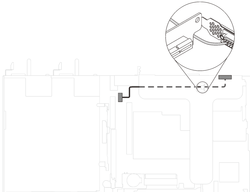
Abbildung 81. Kabelführung für das serielle Anschlussmodul, das im PCIe-Steckplatz 1 installiert ist
