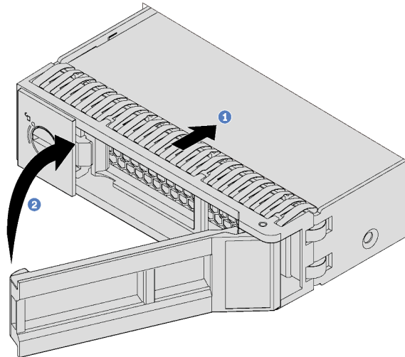
Abbildung 52. Installation eines Simple-Swap-Laufwerks
