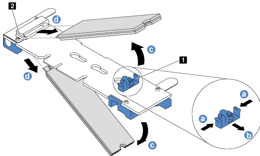
Abbildung 83. Entfernen des M.2-Laufwerks
