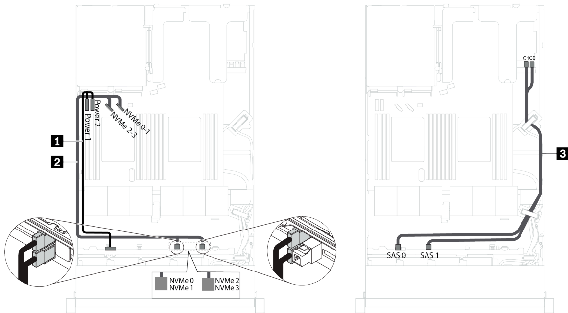
Abbildung 21. Kabelführung für Servermodelle mit sechs 2,5-Zoll-SAS-/SATA-Laufwerken, vier 2,5-Zoll-NVMe-Laufwerken und einem 8i RAID-Adapter
