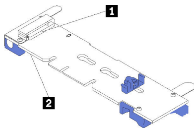
Abbildung 85. M.2-Laufwerksteckplatz
