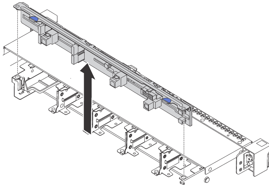
Abbildung 69. Entfernen der Rückwandplatine für zehn 2,5-Zoll-Hot-Swap-Laufwerke
