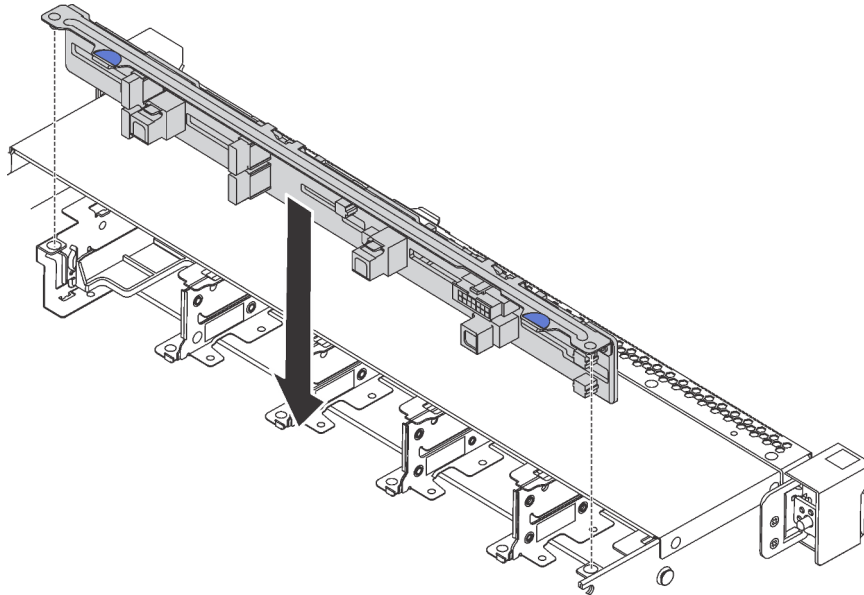
Abbildung 70. Installation einer Rückwandplatine für zehn 2,5-Zoll-Hot-Swap-Laufwerke
