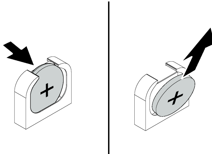
Abbildung 73. Entfernen der CMOS-Batterie
