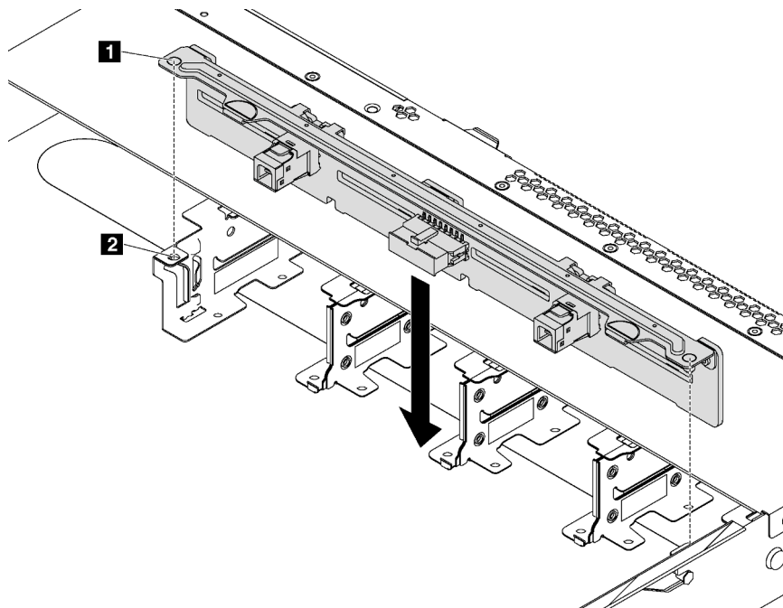
Abbildung 68. Installation einer Rückwandplatine für acht 2,5-Zoll-Hot-Swap-Laufwerke
