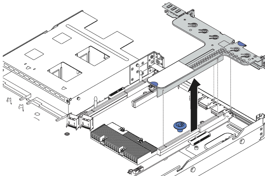
Abbildung 55. Entfernen der Adapterkartenbaugruppe
