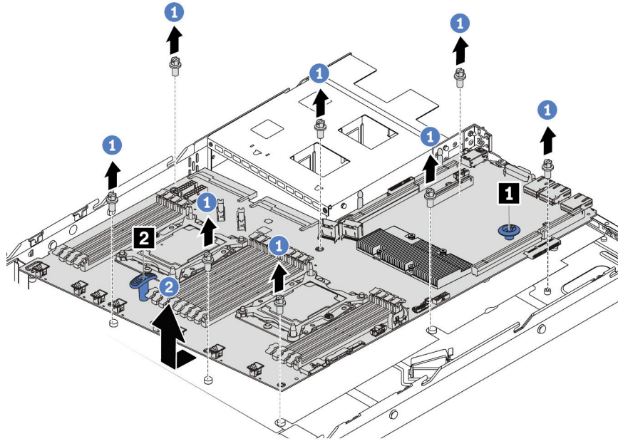
Abbildung 112. Entfernen der Systemplatine
