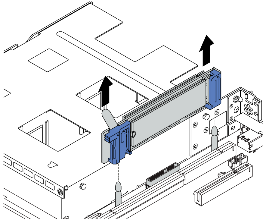
Abbildung 82. Entfernen der M.2-Rückwandplatine
