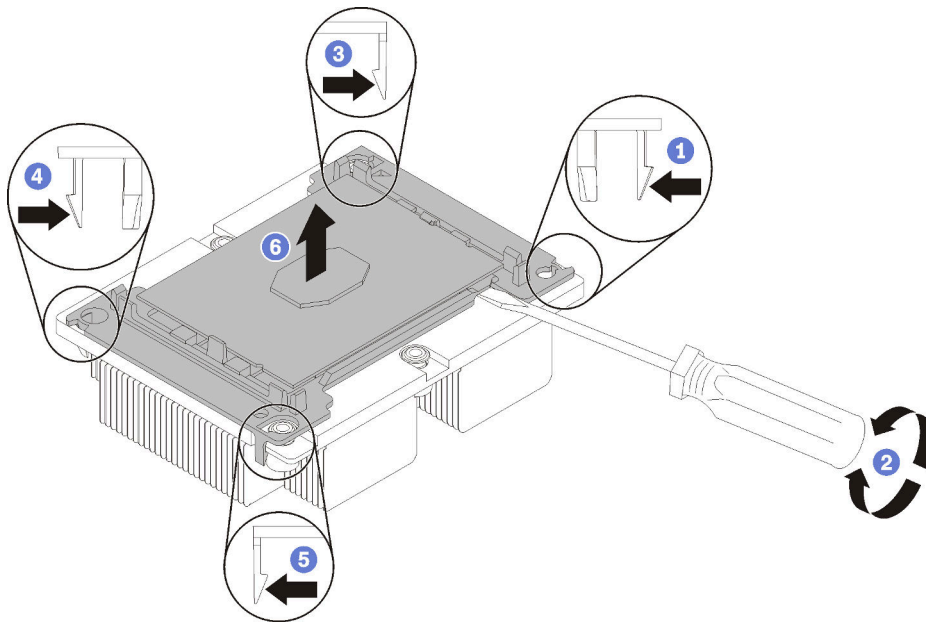
Abbildung 105. Trennen von Kühlkörper und Prozessor
