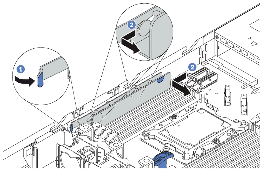
Abbildung 111. Entfernen des Kabelhalters
