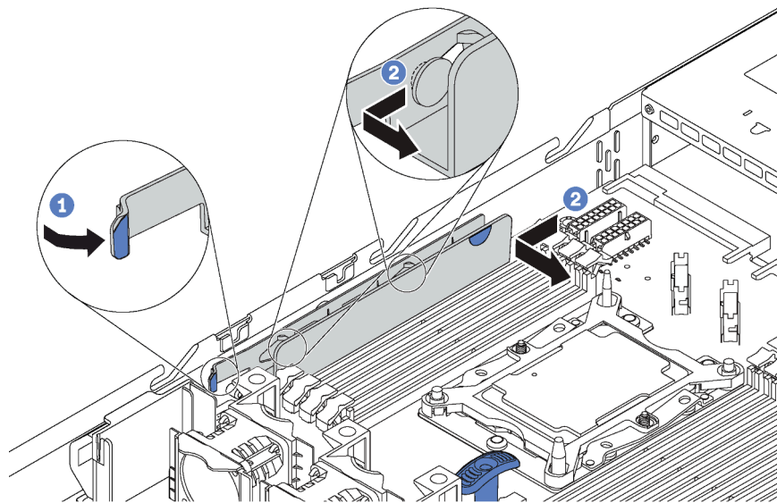
Abbildung 113. Entfernen des Kabelhalters
