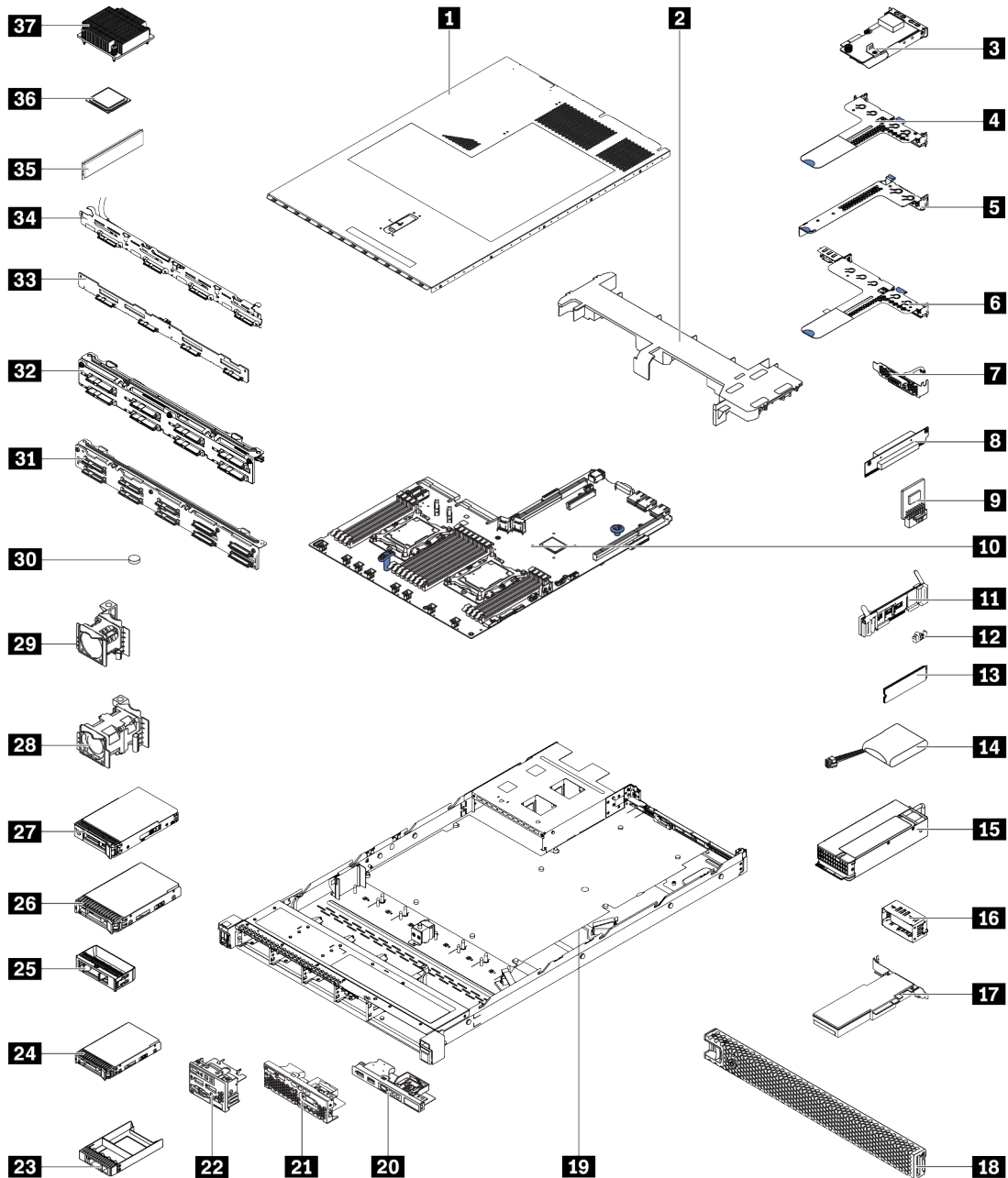
Abbildung 25. Serverkomponenten
