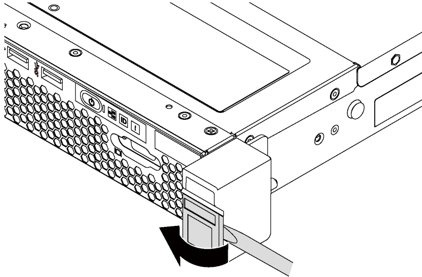
Abbildung 30. Entfernen des Kennungsetikettenschildes
