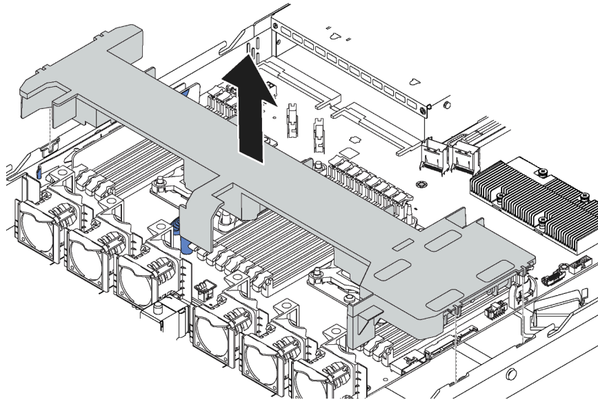
Abbildung 28. Entfernen der Luftführung
