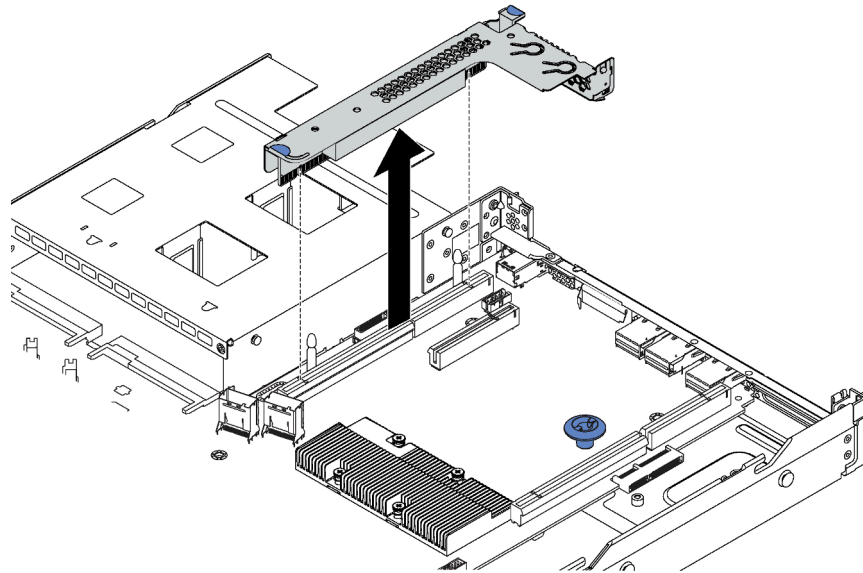
Abbildung 77. Entfernen der Adapterkartenbaugruppe
