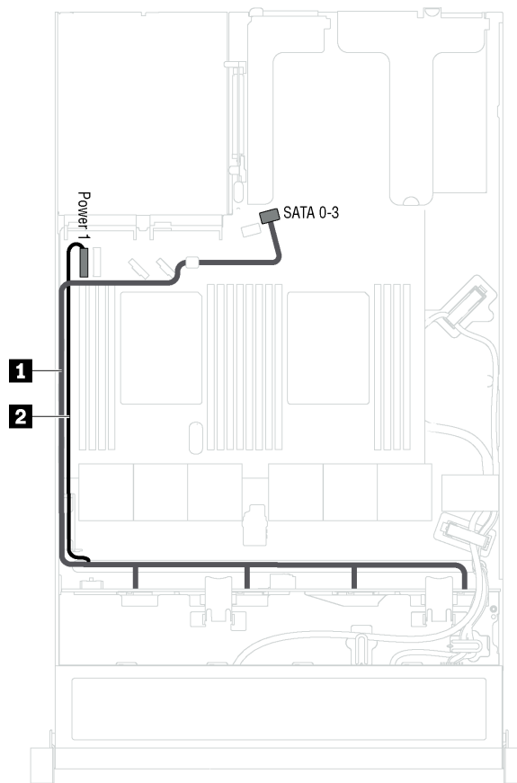
Abbildung 24. Kabelführung für Servermodelle mit vier 3,5-Zoll-Simple-Swap-Laufwerken
