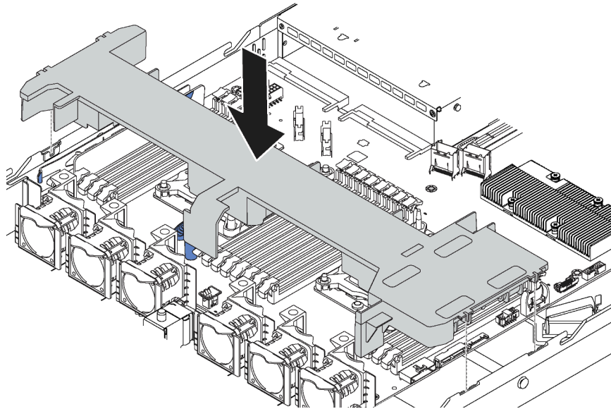
Abbildung 29. Installation der Luftführung
