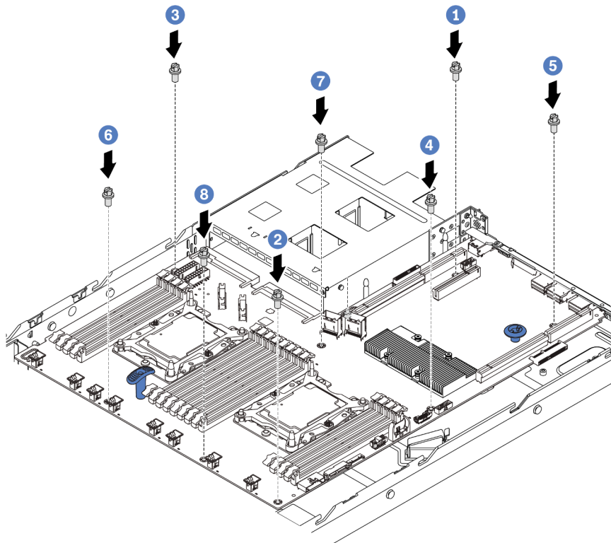
Abbildung 115. Installationsreihenfolge der Schrauben an der Systemplatine
