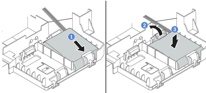
Abbildung 90. Installation des RAID-Superkondensatormoduls
