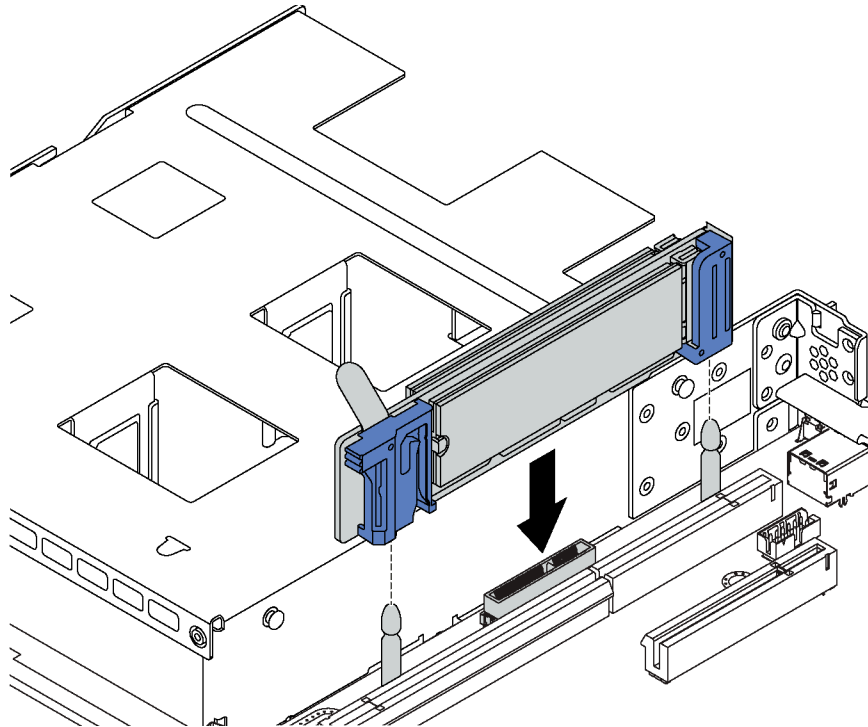
Abbildung 88. Installieren der M.2-Rückwandplatine
