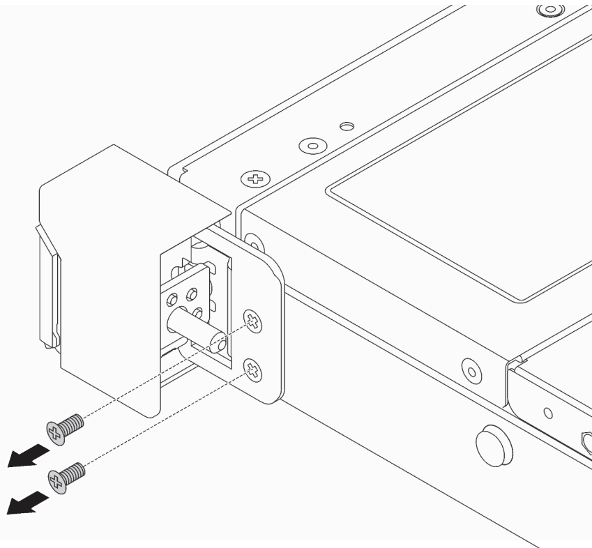
Abbildung 31. Entfernen der Schrauben der Rack-Verriegelung
