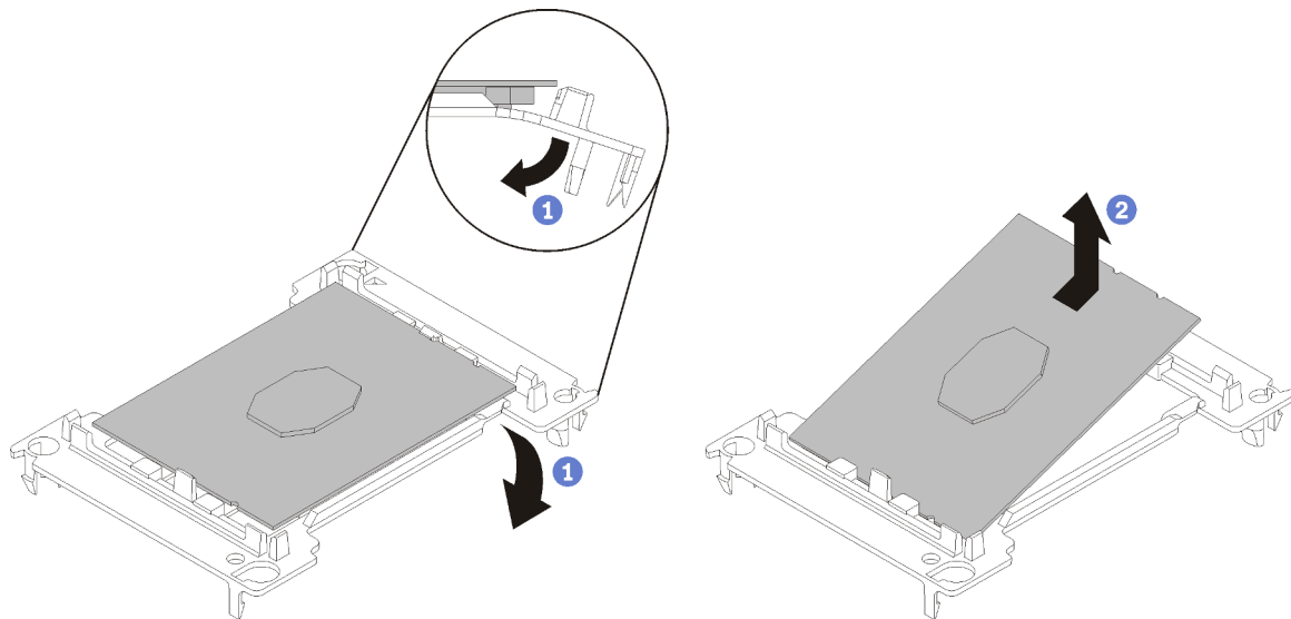
Abbildung 106. Halterung für einen Prozessor entfernen
