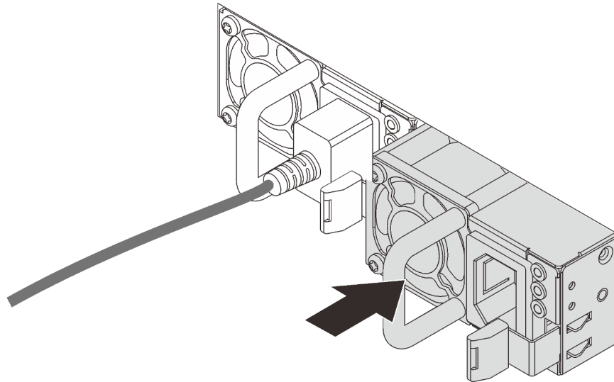
Abbildung 103. Installation des Hot-Swap-Netzteils
