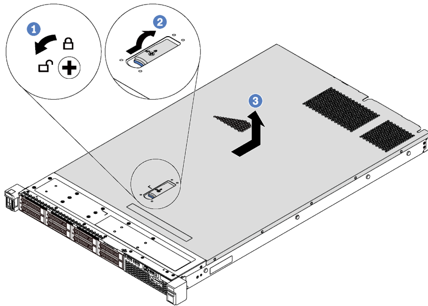
Abbildung 26. Entfernen der oberen Abdeckung
