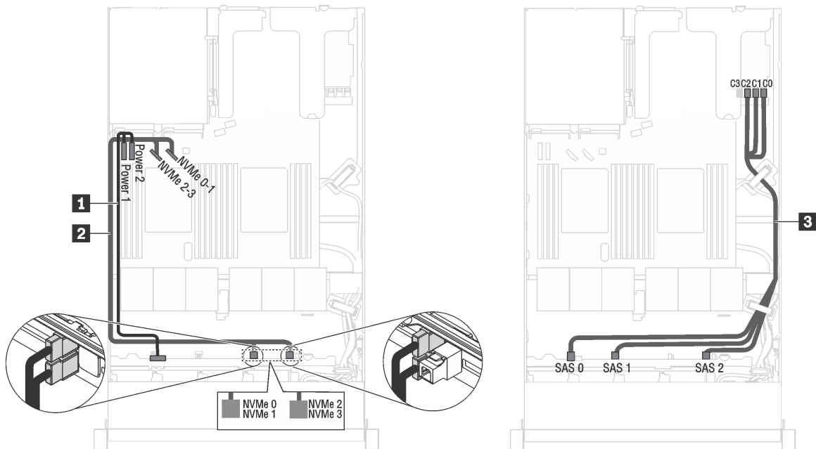
Abbildung 20. Kabelführung für Servermodelle mit sechs 2,5-Zoll-SAS-/SATA-Laufwerken, vier 2,5-Zoll-SAS-/SATA-/NVMe-Laufwerken und einem 16i RAID-Adapter
