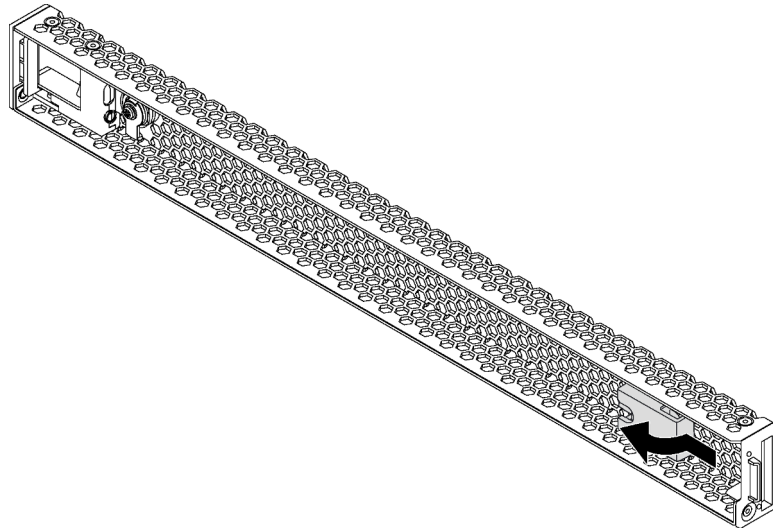
Abbildung 38. Schlüssel entfernen
