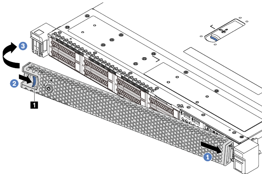
Abbildung 39. Installation der Sicherheitsfrontblende
