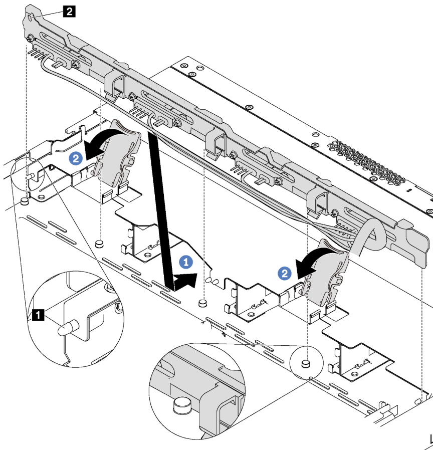
Abbildung 72. Rückwandbaugruppe für Simple-Swap-Laufwerke installieren
