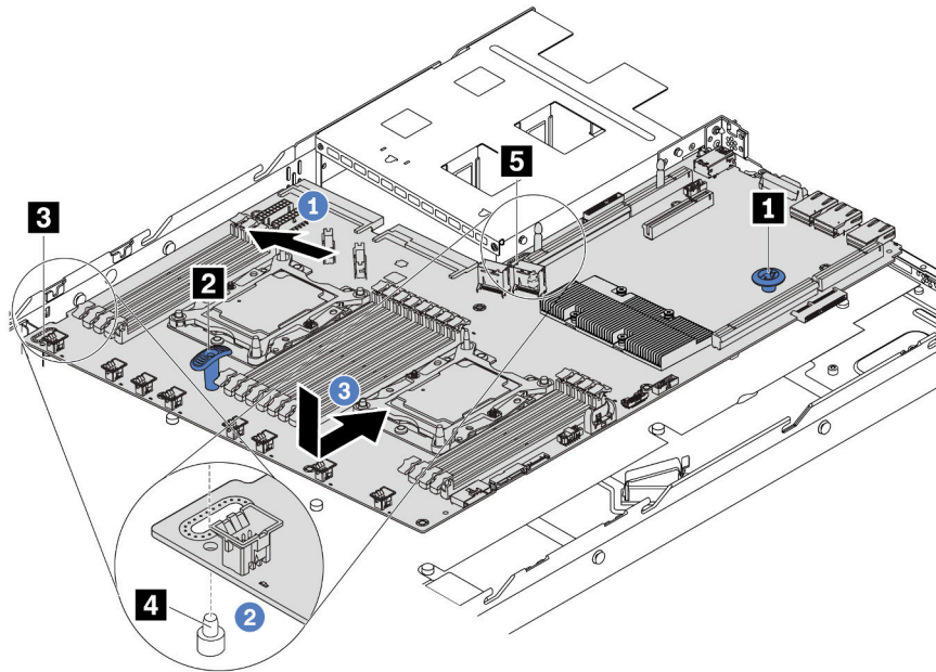
Abbildung 114. Systemplatineeinbau
