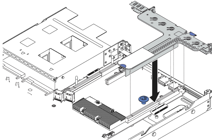
Abbildung 58. Installation der Adapterkartenbaugruppe
