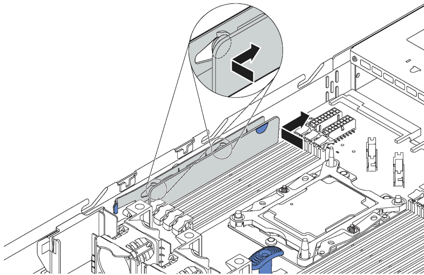
Abbildung 116. Installation des Kabelhalters
