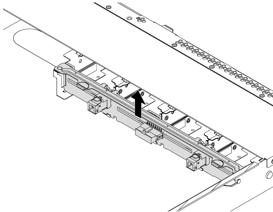
Abbildung 67. Entfernen der Rückwandplatine für acht 2,5-Zoll-Hot-Swap-Laufwerke
