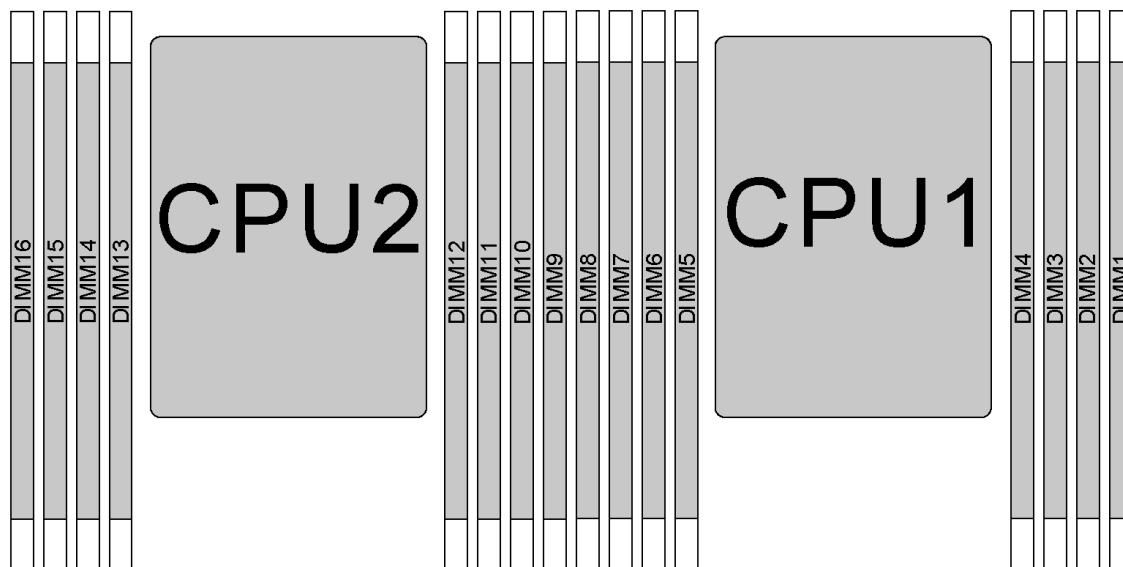
Abbildung 45. DIMM-Positionen
