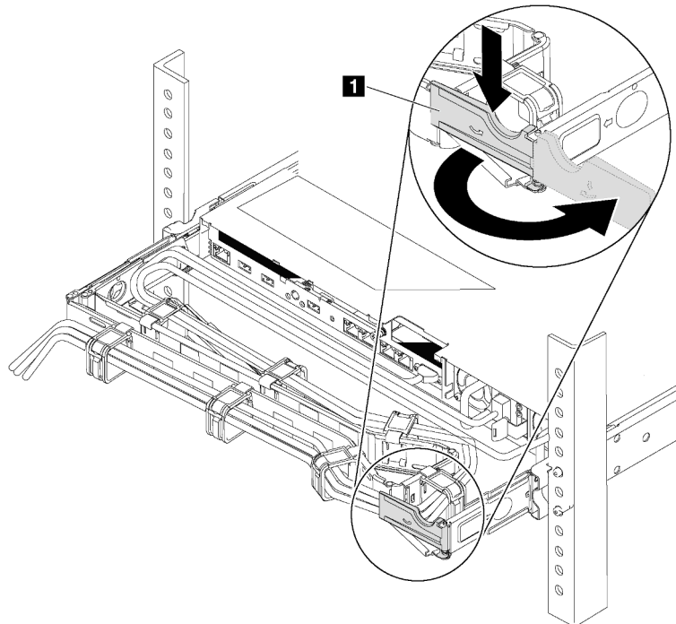
Abbildung 98. CMA-Anpassung
