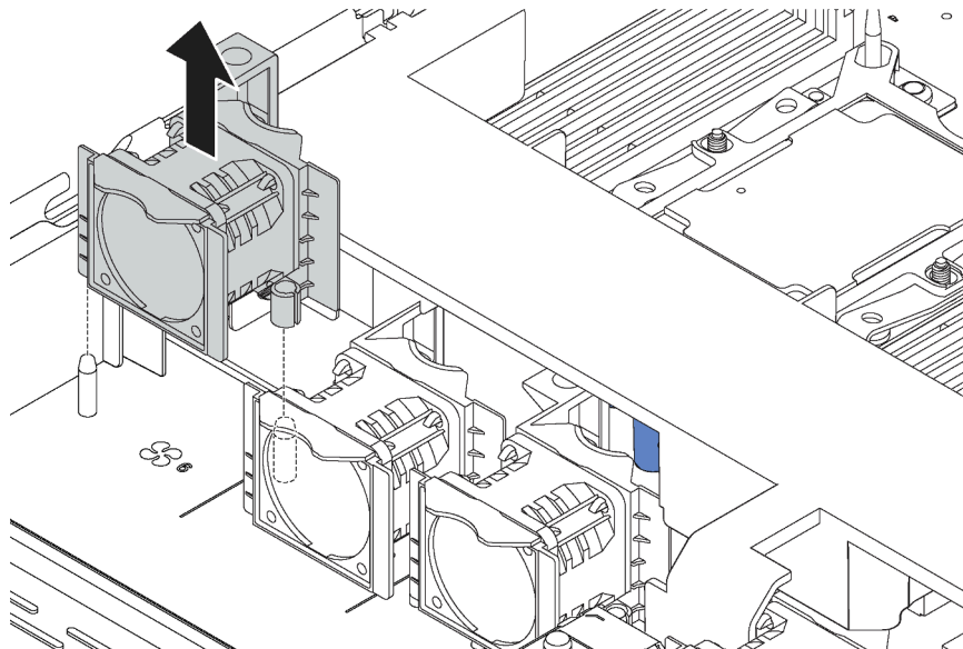
Abbildung 41. Entfernen des Systemlüfters
