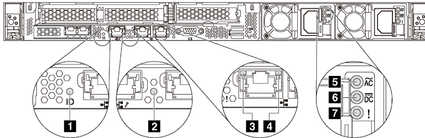
Abbildung 10. Anzeigen an der Rückseite
