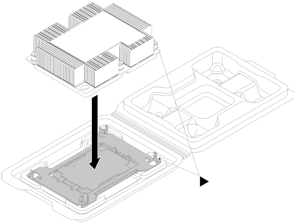
Abbildung 109. Zusammensetzen des PHM im Versandeinbaurahmen
