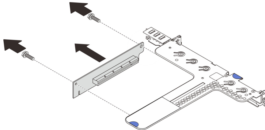
Abbildung 56. Ausbau der Adapterkarte
