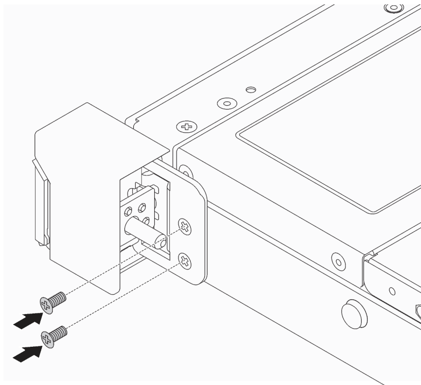
Abbildung 34. Einsetzen der Schrauben der Rack-Verriegelung
