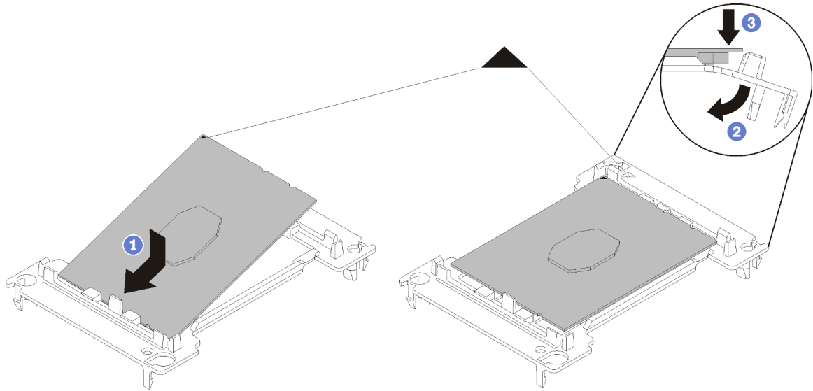
Abbildung 107. Halterung für einen Prozessor installieren
