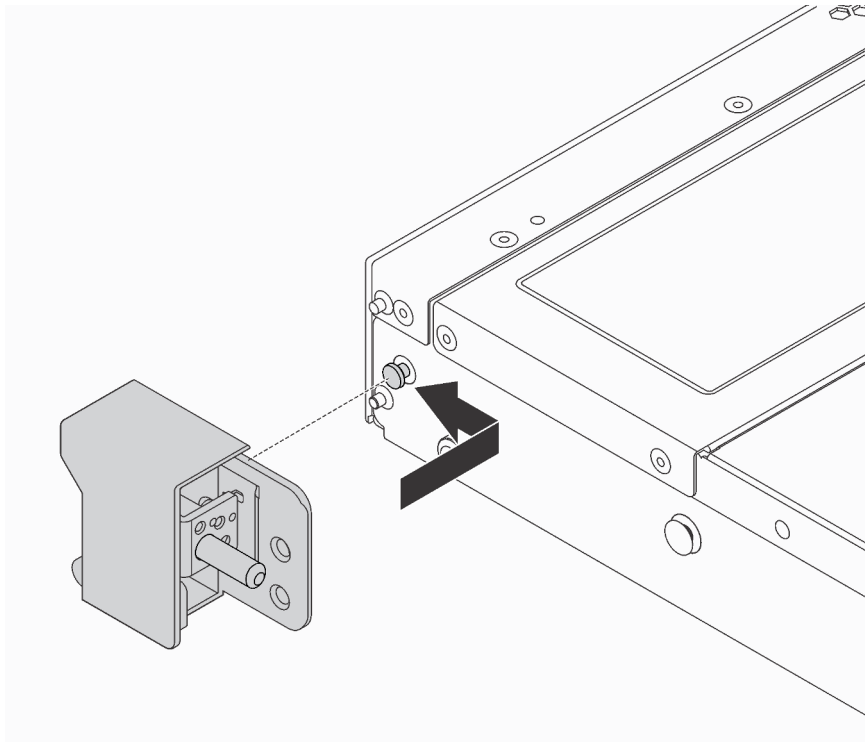
Abbildung 33. Installation der Rack-Verriegelung
