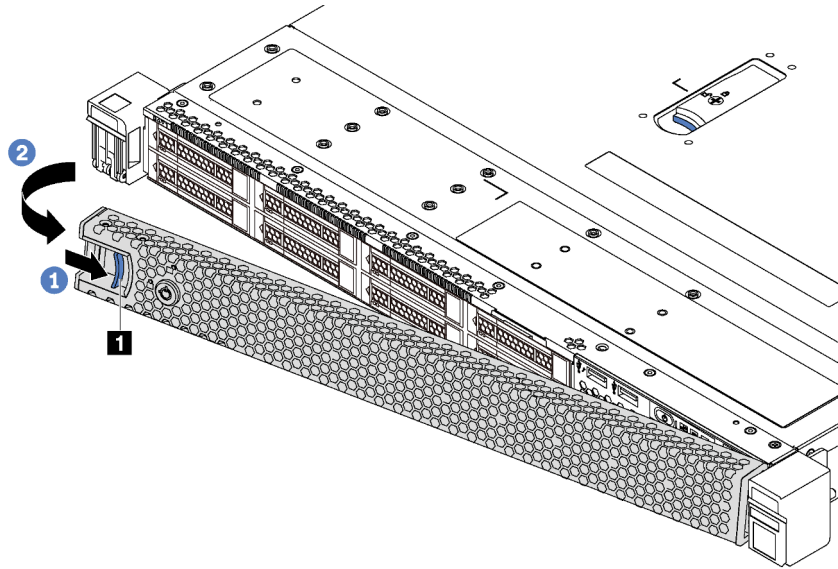
Abbildung 37. Entfernen der Sicherheitsfrontblende
