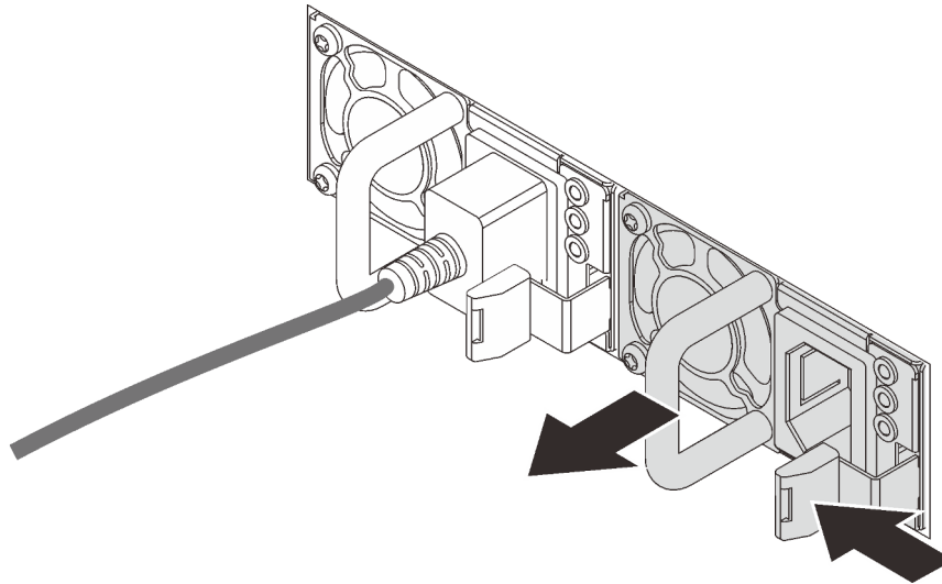
Abbildung 99. Entfernen des Hot-Swap-Netzteils
