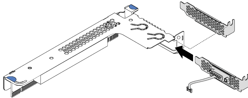
Abbildung 80. Installation des seriellen Anschlussmoduls
