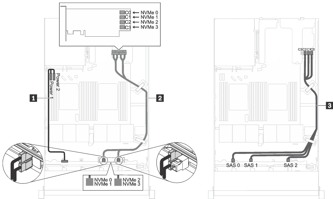
Abbildung 22. Kabelführung für Servermodelle mit sechs 2,5-Zoll-SAS/SATA-Laufwerken, vier 2,5-Zoll-NVMe-Laufwerken, einem 16i-RAID-Adapter im PCIe-Steckplatz 1 und einem 1610-4P-NVMe-Switch-Adapter im PCIe-Steckplatz 2
