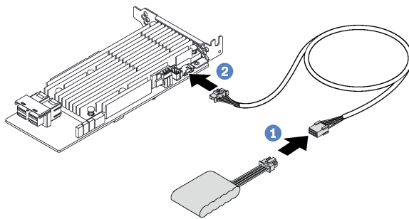
그림 12. RAID 슈퍼 캐패시터 모듈과 RAID 어댑터의 연결
