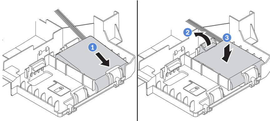
그림 48. RAID 슈퍼 커패시터 모듈의 설치
