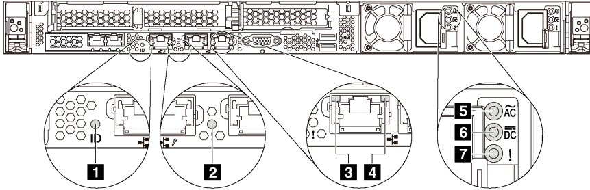
그림 10. 뒷면 LED
