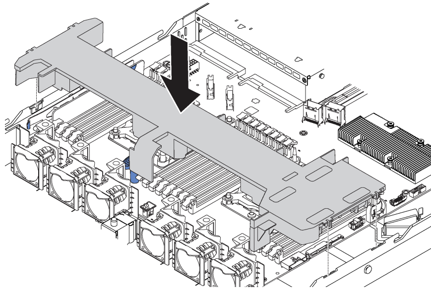
그림 49. 공기 조절 장치 설치
