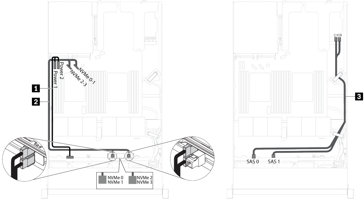
그림 19. 2.5인치 SAS/SATA 드라이브 6개, 2.5인치 NVMe 드라이브 4개, 8i RAID 어댑터 1개가 지원되는 서버 모델의 케이블 배선
