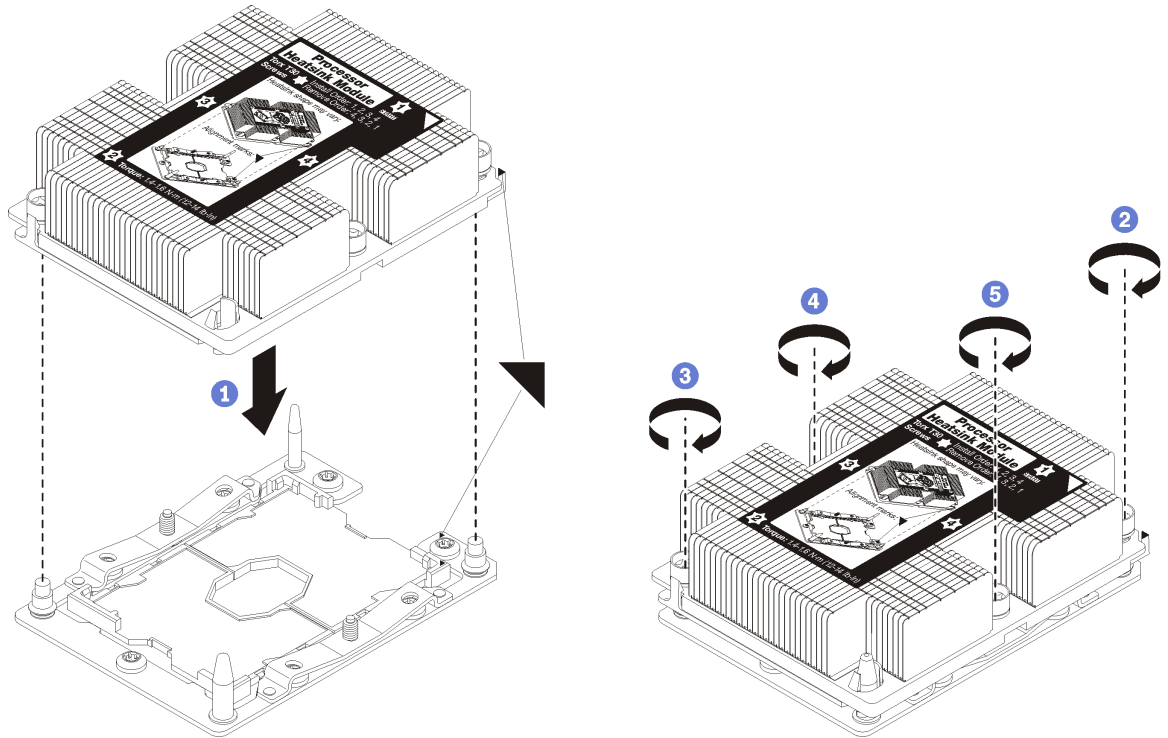
그림 28. PHM 설치
