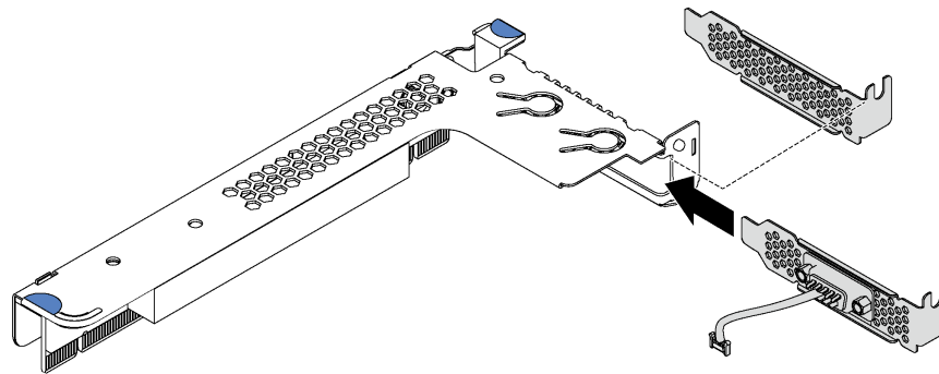
그림 46. 직렬 포트 모듈 설치
