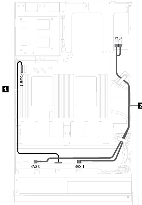
그림 16. 8개의 2.5인치 핫 스왑 드라이브가 지원되는 서버 모델의 케이블 배선
