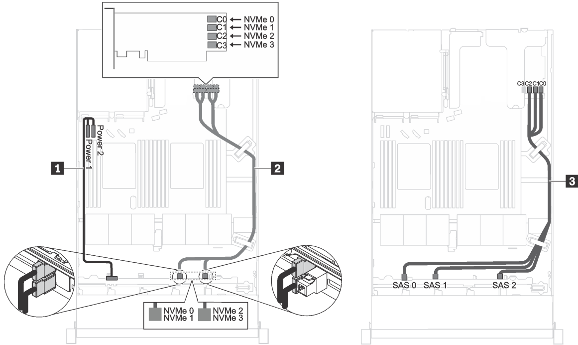
그림 20. PCIe 슬롯 2에 2.5인치 SAS/SATA 드라이브 6개, 2.5인치 NVMe 드라이브 4개, PCIe 슬롯 1의 16i RAID 어댑터 1개 및 1610-4P NVMe 스위치 어댑터 1개가 지원되는 서버 모델
