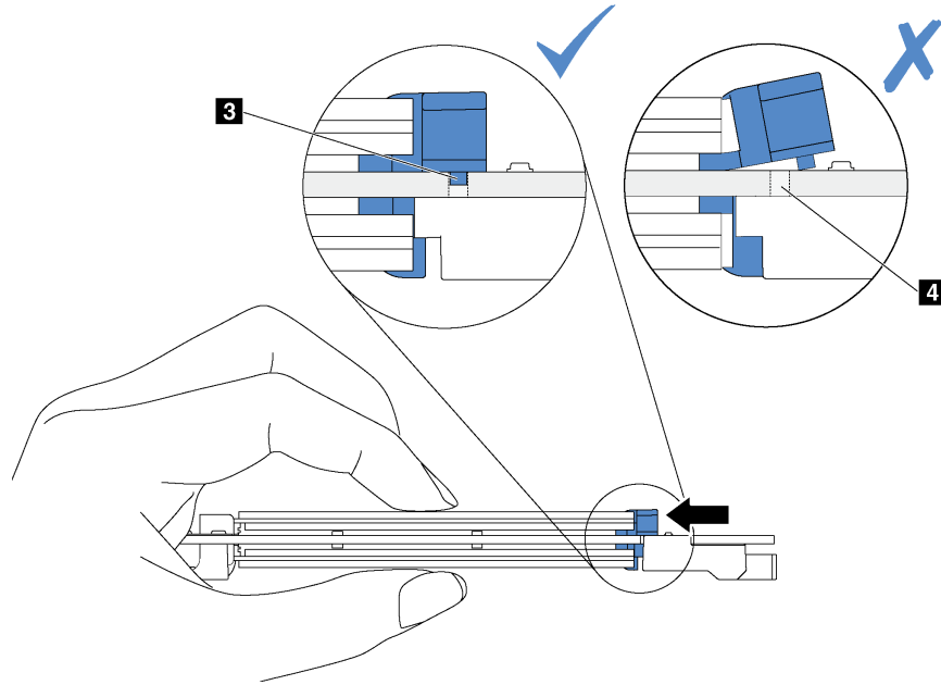
그림 34. 고정장치를 미는 방법
