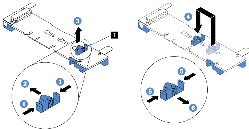
그림 36. M.2 고정장치 조정
