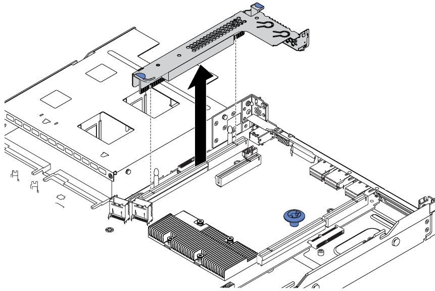
그림 45. 라이저 어셈블리 제거
