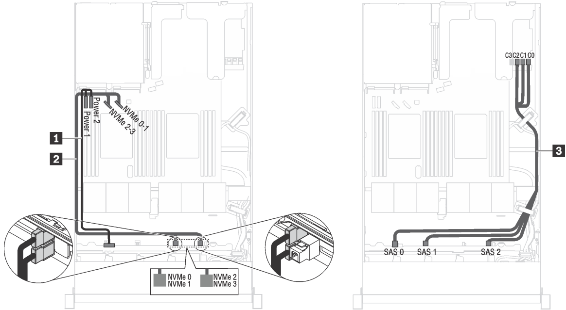
그림 18. 2.5인치 SAS/SATA 드라이브 6개, 2.5인치 SAS/SATA/NVMe 드라이브 4개 및 16i RAID 어댑터 1개 장착 서버 모델의 케이블 배선
