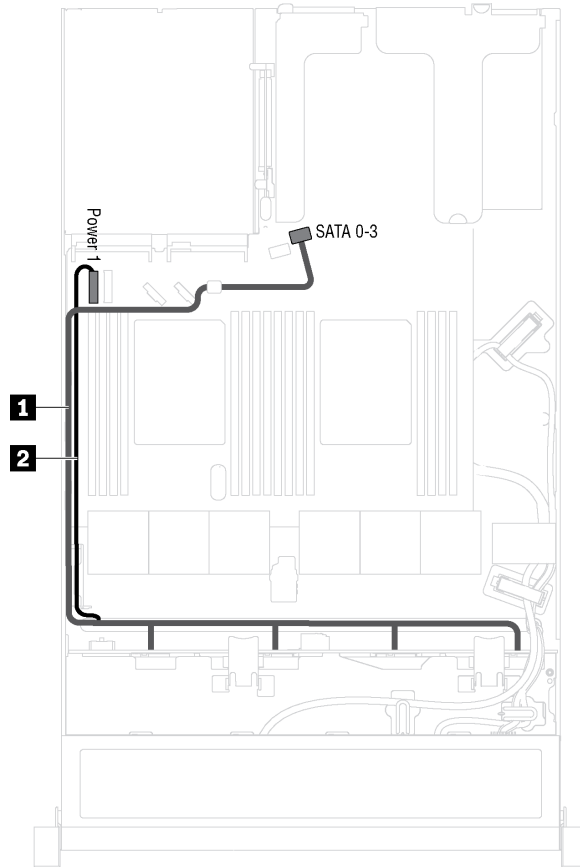
그림 22. 4개의 3.5인치 심플 스왑 드라이브가 있는 서버 모델의 케이블 배선
