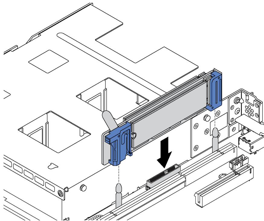
그림 35. M.2 백플레인 설치
