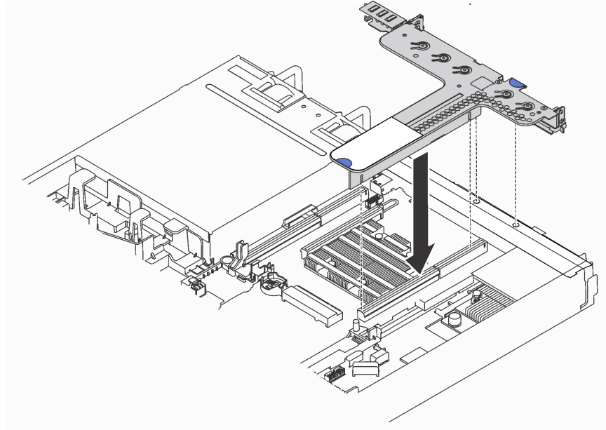
그림 44. 라이저 어셈블리 설치
