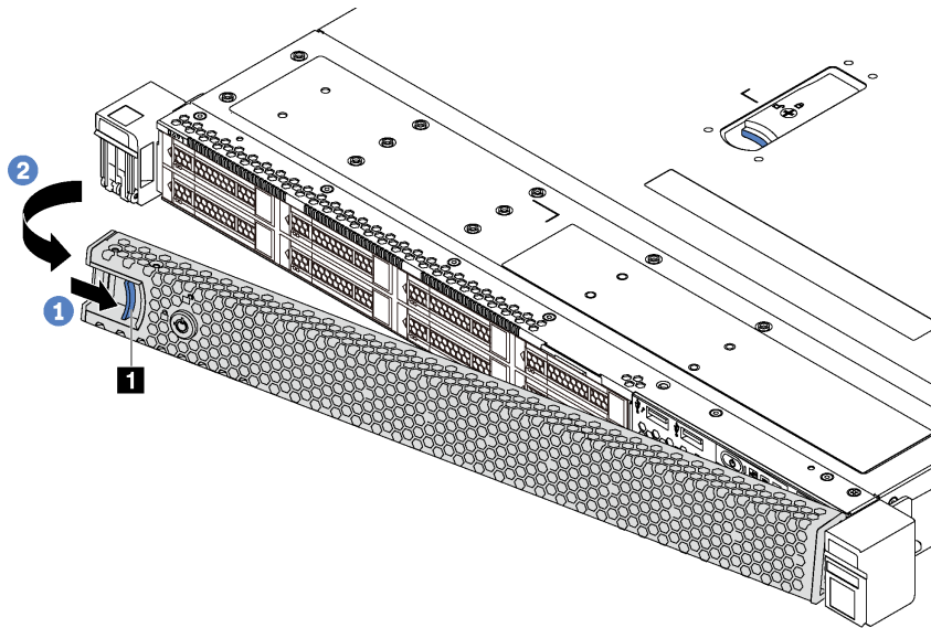
그림 25. 보안 베젤 제거
