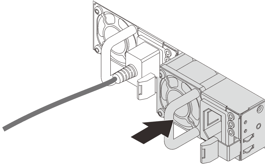
그림 39. 핫 스왑 전원 공급 장치 설치
