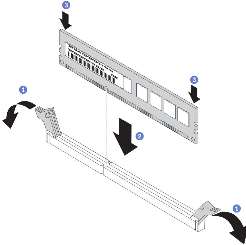
그림 30. 메모리 모듈 설치
