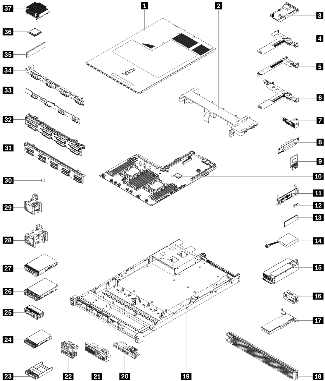
그림 23. 서버 구성 요소
