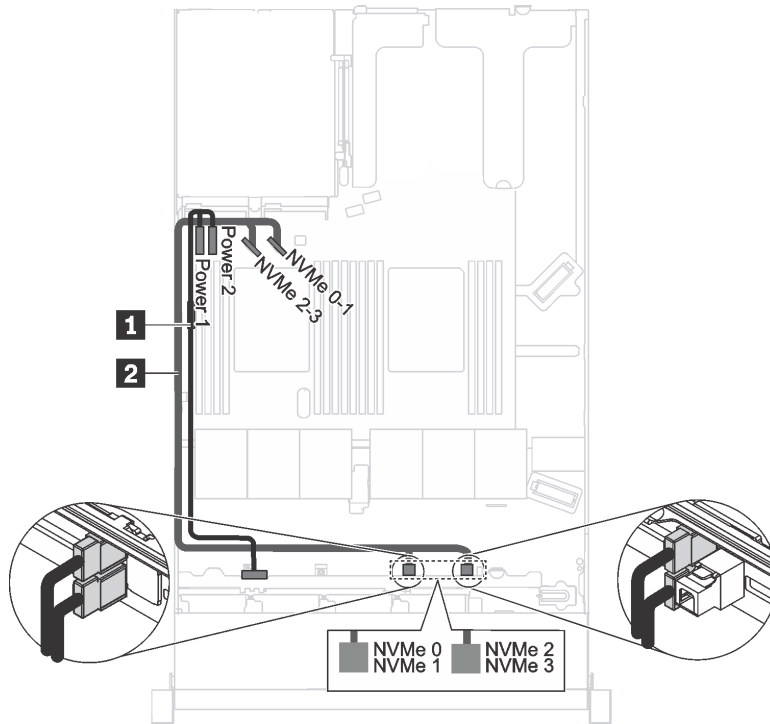
그림 21. 2.5인치 NVMe 드라이브 4개가 지원되고 RAID 어댑터가 지원되지 않는 서버 모델의 케이블 배선
