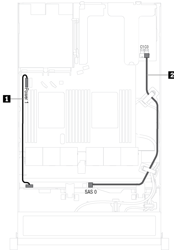
그림 14. 4개의 3.5인치 핫 스왑 드라이브가 장착된 서버 모델에 대한 케이블 배선
