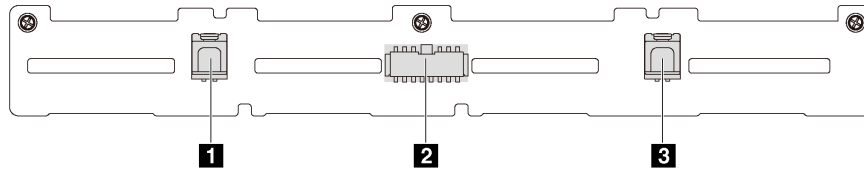
그림 15. 8개의 2.5인치 핫 스왑 드라이브용 백플레인의 커넥터
