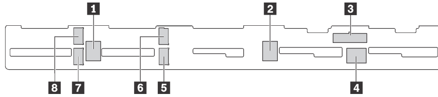
그림 17. 10개의 2.5인치 핫 스왑 드라이브용 백플레인의 커넥터
