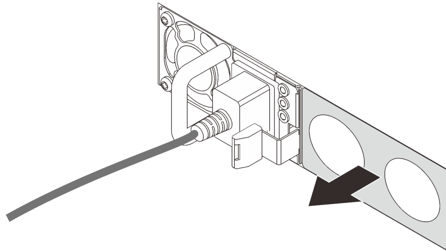
그림 38. 핫 스왑 전원 공급 장치 필터 제거
