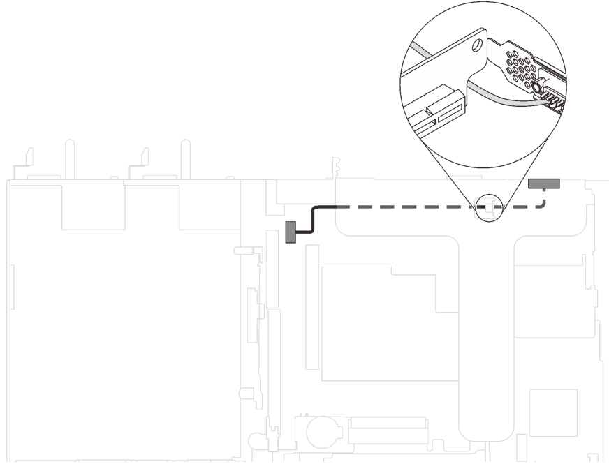
그림 47. PCIe 슬롯 10에 설치된 직렬 포트 모듈의 케이블 라우팅
