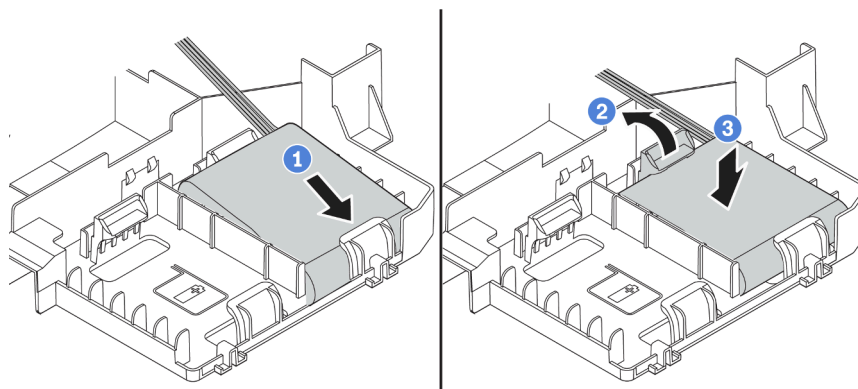
Figura 48. Instalação de um módulo de supercapacitor RAID
