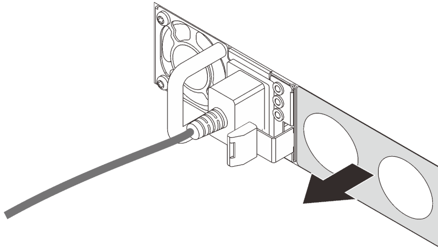
Figura 38. Remoção do preenchimento da fonte de alimentação hot-swap
