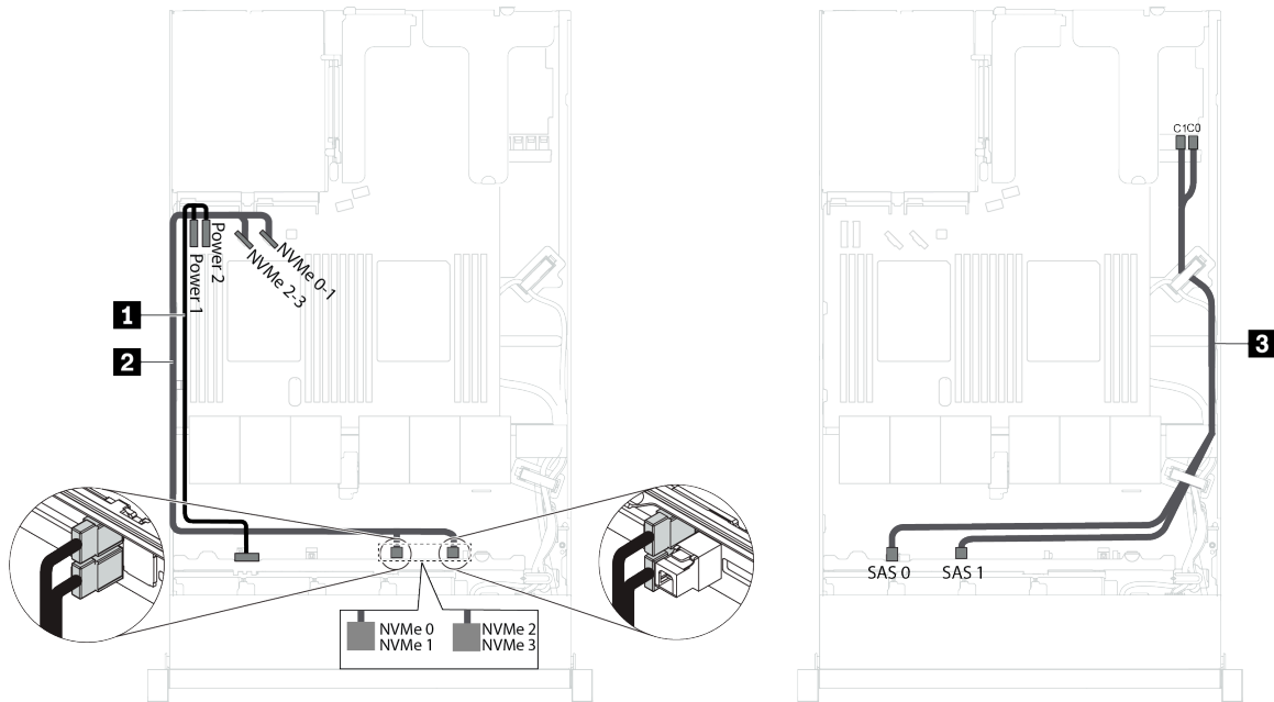
Figura 19. Roteamento de cabos para modelos de servidor com seis unidades SAS/SATA de 2,5 polegadas, quatro unidades NVMe de 2,5 polegadas e um adaptador RAID 8i
