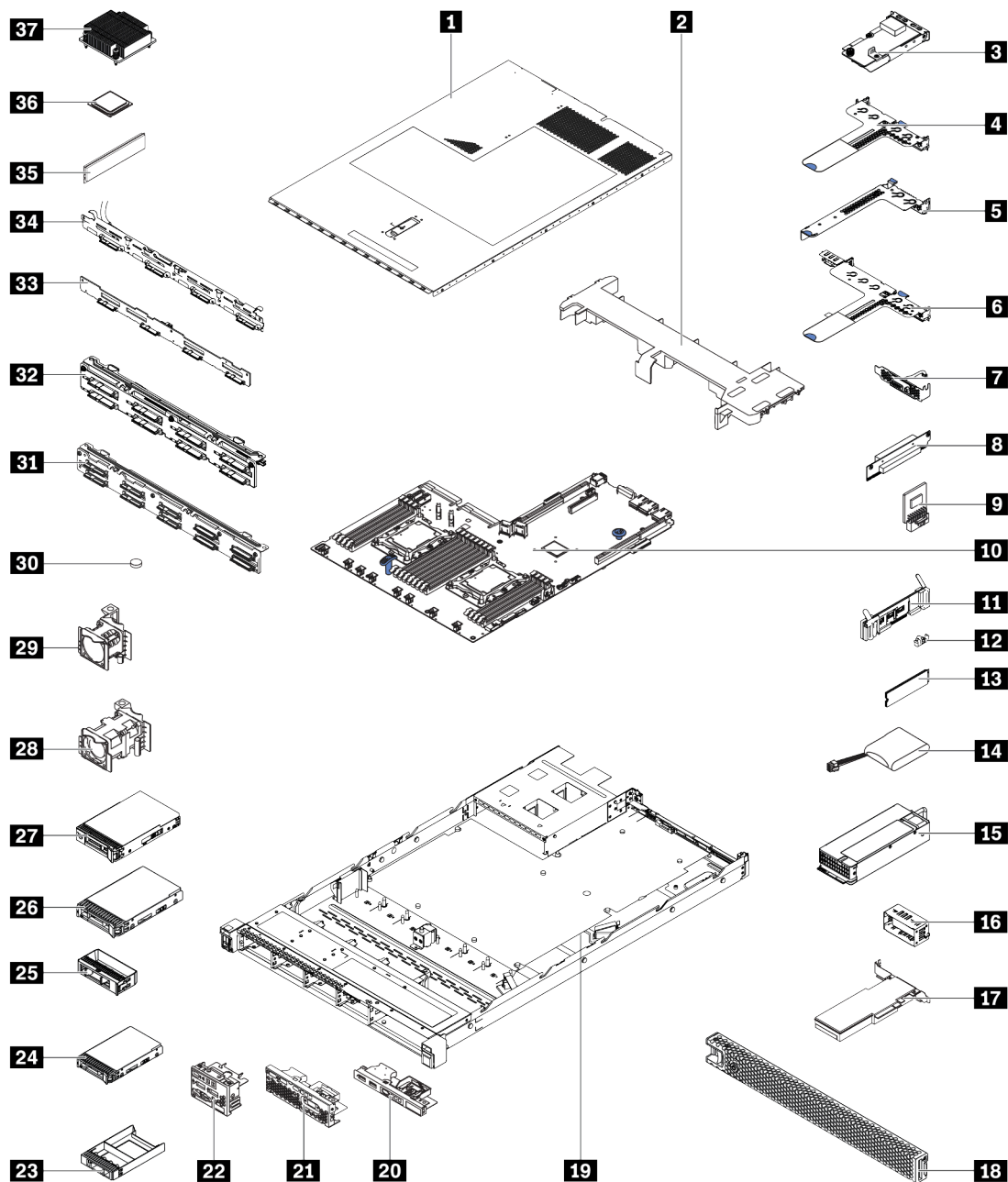
Figura 23. Componentes do servidor
