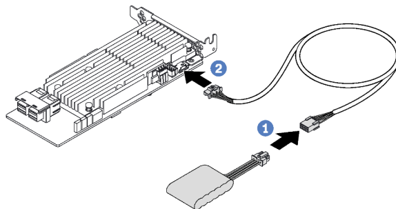
Figura 12. Conectando o módulo de supercapacitor RAID ao adaptador RAID
