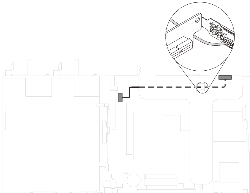
Figura 47. Roteamento de cabos do módulo de porta serial instalado no slot PCIe 1
