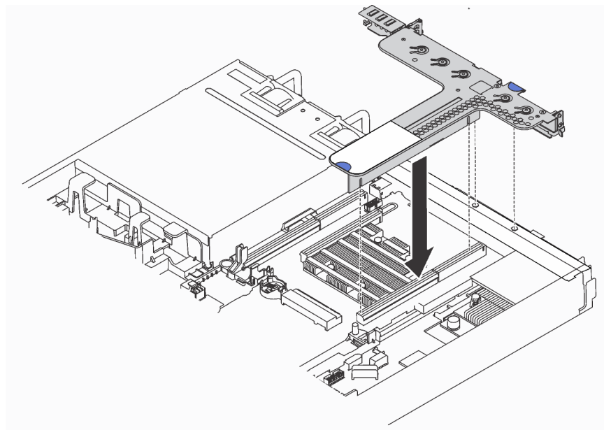
Figura 44. Instalação do conjunto de placa riser
