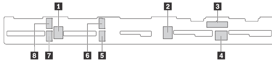
Figura 17. Conectores no backplane para dez unidades hot-swap de 2,5 polegadas
