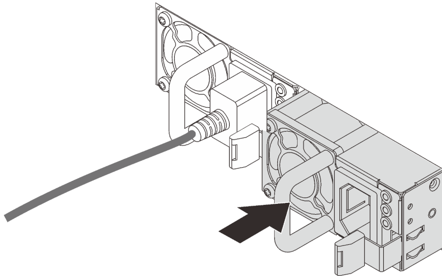
Figura 39. Instalação da fonte de alimentação hot-swap
