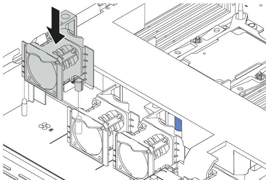
Figura 29. Instalação do ventilador do sistema
