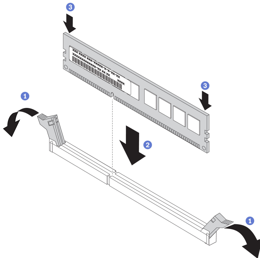
Figura 30. Instalação do módulo de memória
