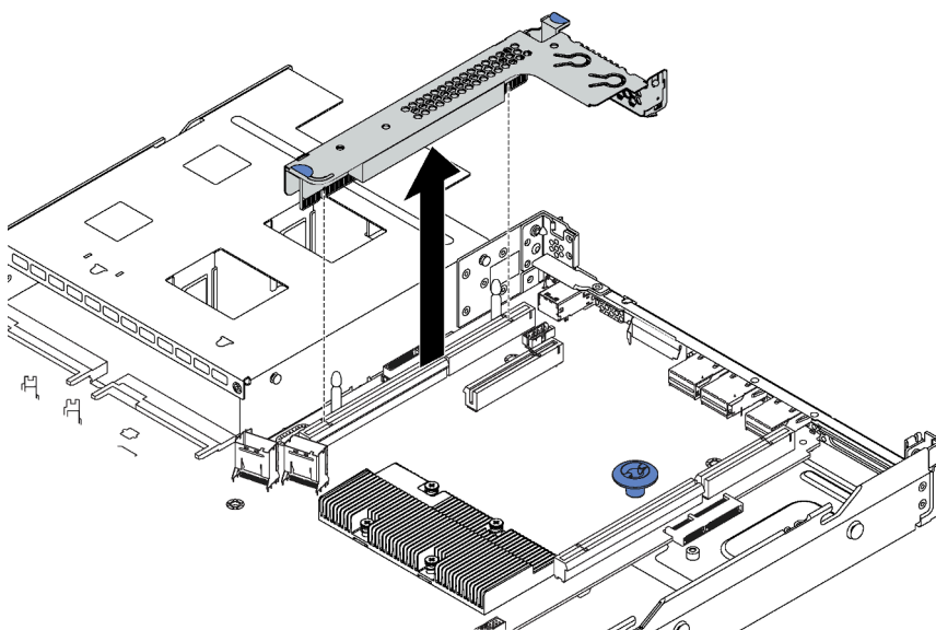
Figura 45. Remoção do conjunto da placa riser
