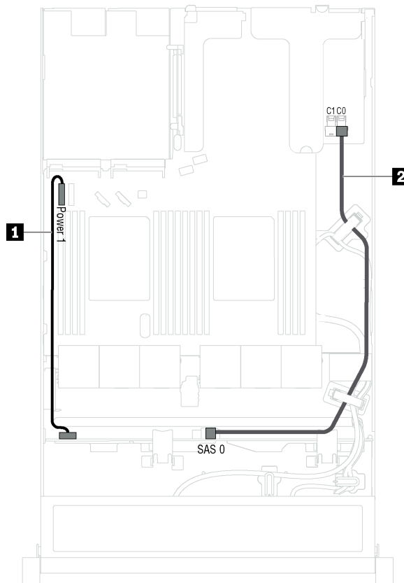
Figura 14. Roteamento de cabos para modelos de servidor com quatro unidades hot-swap de 3,5 polegadas
