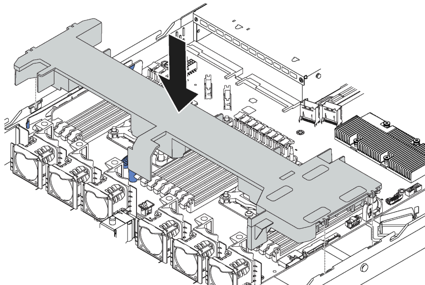
Figura 49. Instalação do defletor de ar
