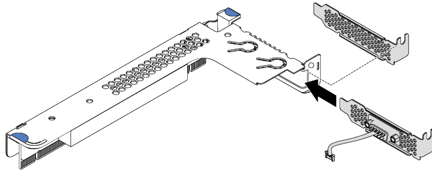
Figura 46. Instalação do módulo de porta serial
