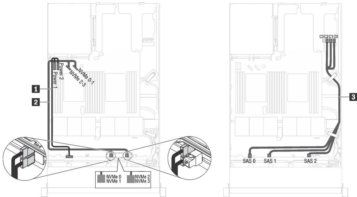
Figura 18. Roteamento de cabos para modelos de servidor com seis unidades SAS/SATA de 2,5 polegadas, quatro unidades SAS/SATA/NVMe de 2,5 polegadas e um adaptador RAID 16i
