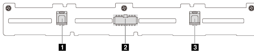
Figura 15. Conectores no painel traseiro para oito unidades hot-swap de 2,5 pol.
