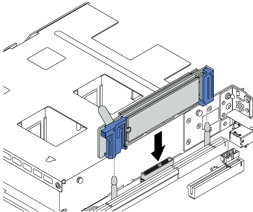
Figura 35. Instalação do backplane M.2
