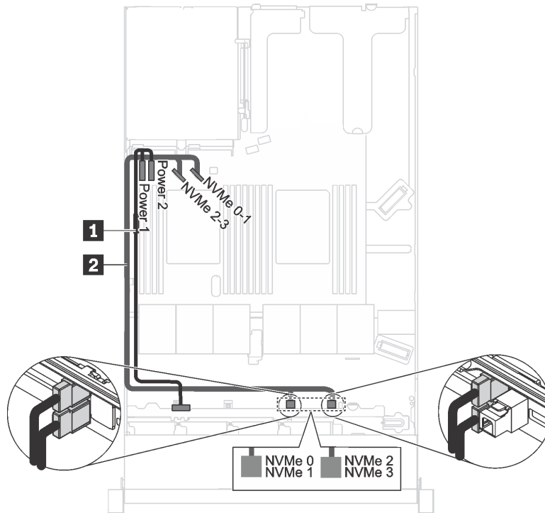
Figura 21. Roteamento de cabos para modelos de servidor com quatro unidades NVMe de 2,5 polegadas e nenhum adaptador RAID
