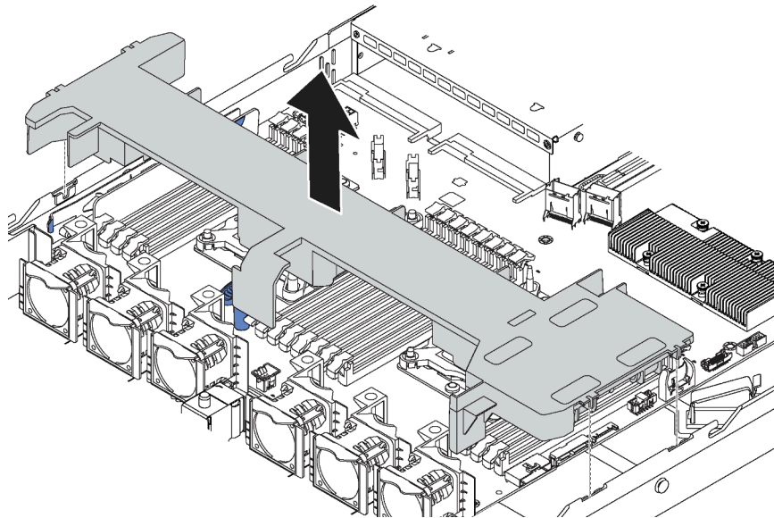
Figura 27. Remoção do defletor de ar
