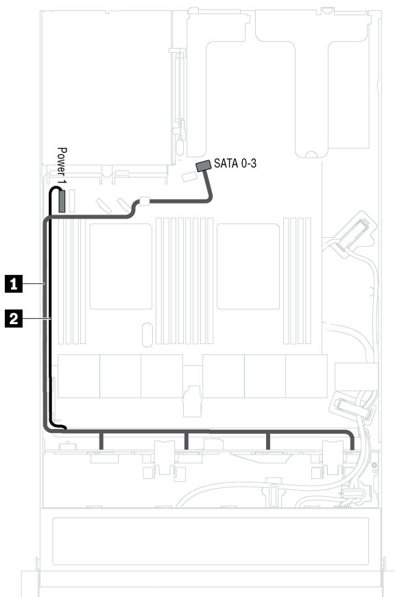
Figura 22. Roteamento de cabos de modelos de servidor com quatro unidades simple-swap de 3,5 polegadas
