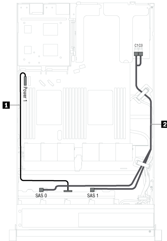
Figura 16. Roteamento de cabos para modelos de servidor com oito unidades hot-swap de 2,5 polegadas
