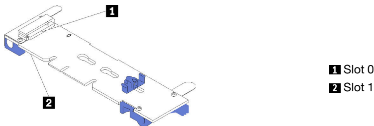
Figura 32. Slot da unidade M.2
