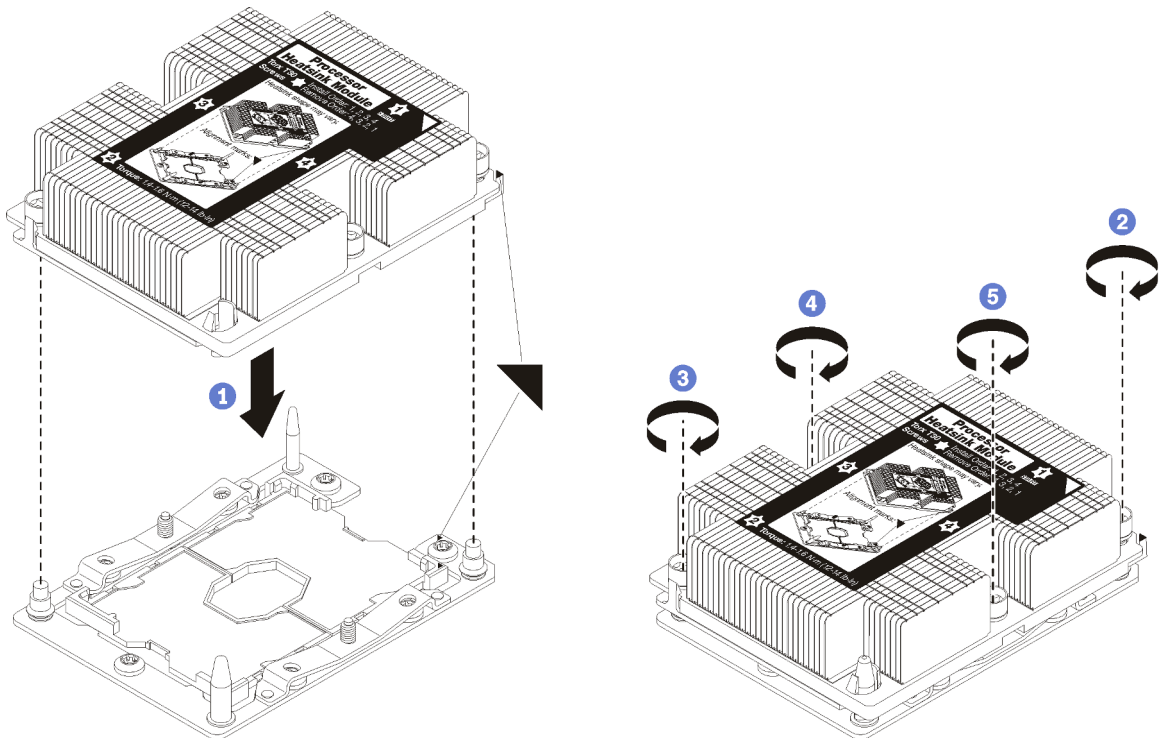
Figura 28. Instalando um PHM
