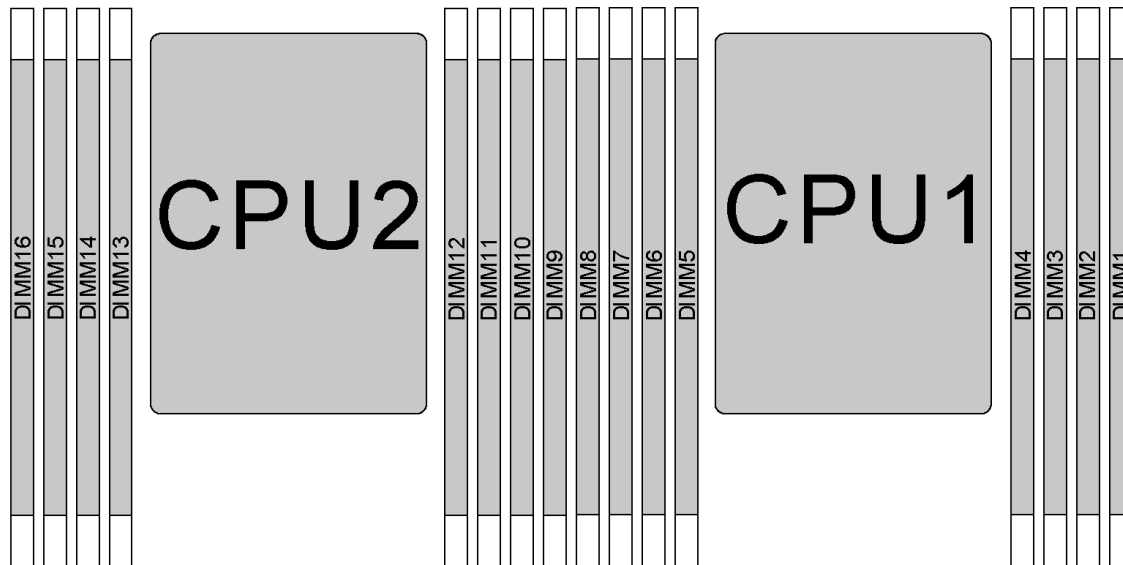
Figura 31. Locais do DIMM
