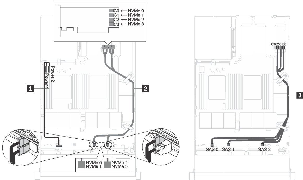
Figura 20. Roteamento de cabos para modelos de servidor com seis unidades SAS/SATA de 2,5 polegadas, quatro unidades NVMe de 2,5 polegadas, um adaptador RAID 16i no slot PCIe 1 e um adaptador de comutador NVMe 1610-4P no slot PCIe 2
