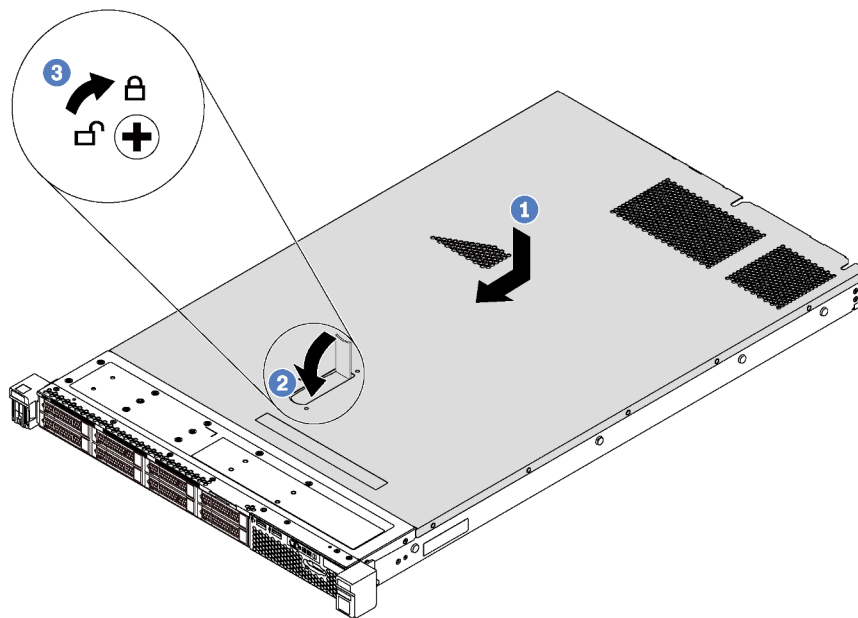
Figura 50. Instalação da tampa superior
