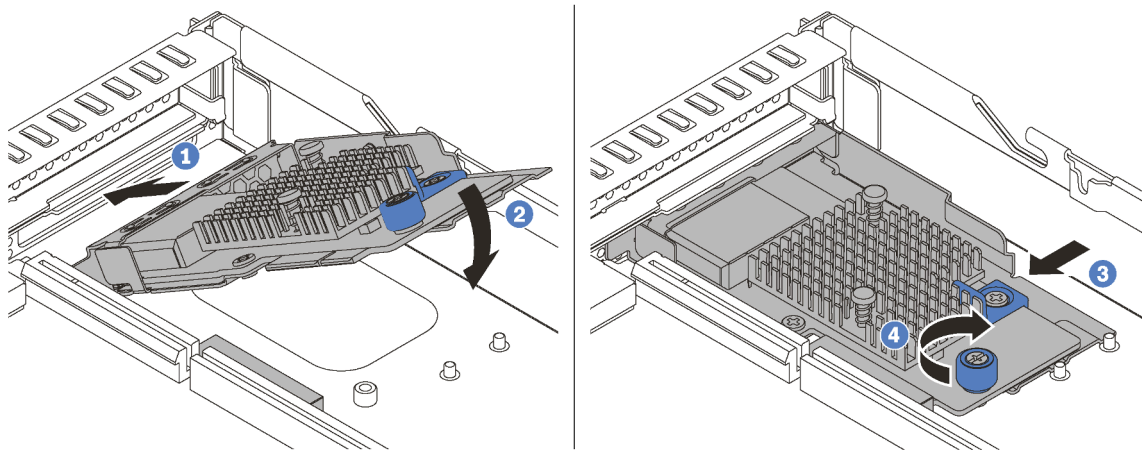
Figura 40. Instalação do adaptador LOM
