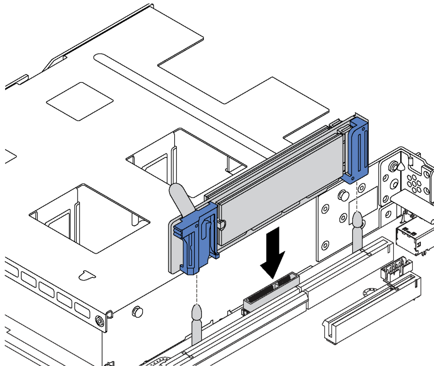
图 35. 安装 M.2 背板
