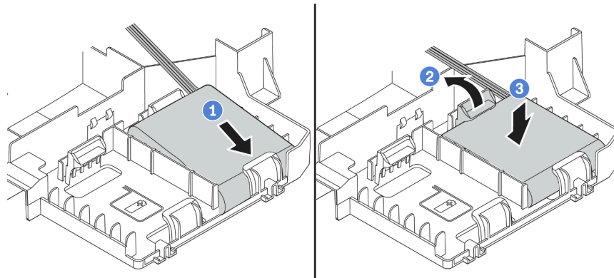
图 48. 安装 RAID 超级电容器模块
