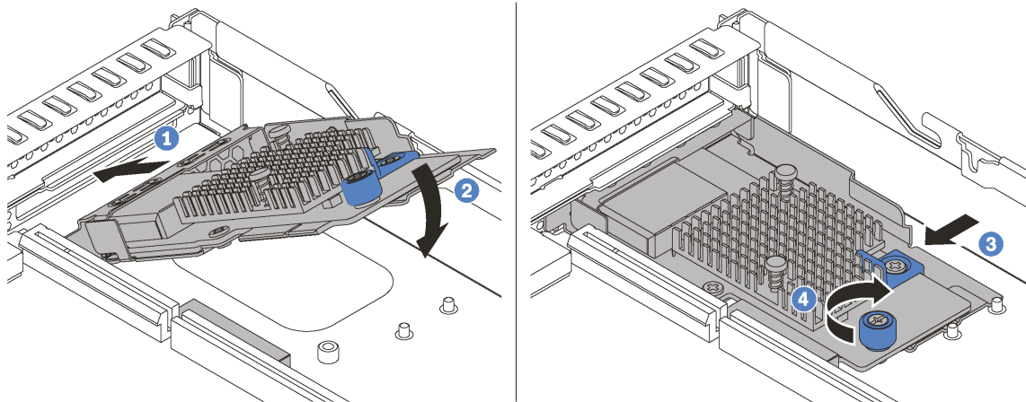
图 40. 安装 LOM 适配器
