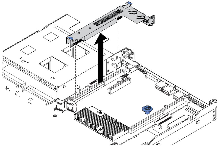
图 45. 卸下转接卡组合件
