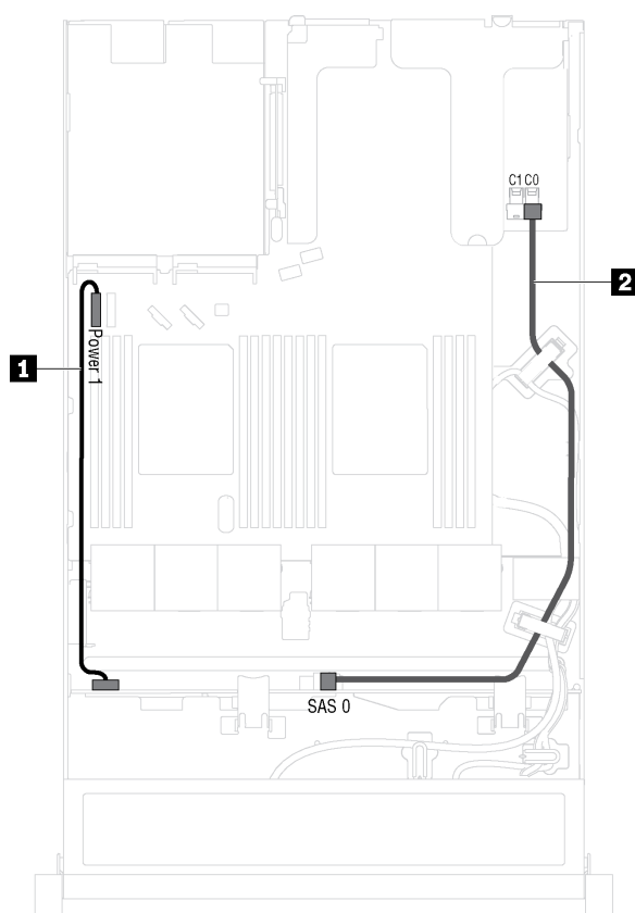
图 14. 配备四个 3.5 英寸热插拔硬盘的服务器型号的线缆布放
