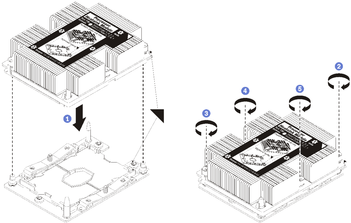
图 28. 安装 PHM
