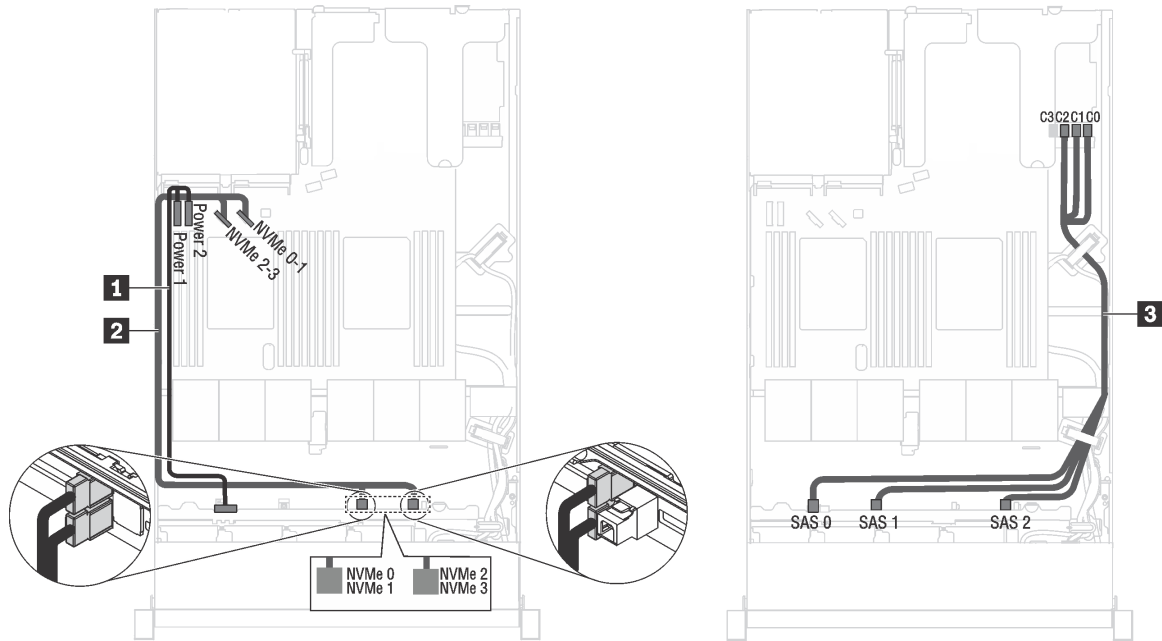
图 18. 配备六个 2.5 英寸 SAS/SATA 硬盘、四个 2.5 英寸 SAS/SATA/NVMe 硬盘和一个 16i RAID 适配器的服务器型号的线缆布放
