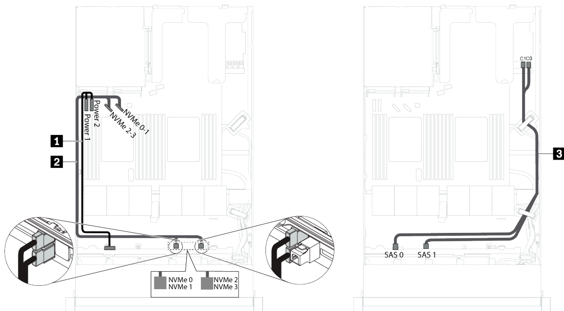
图 19. 配备六个 2.5 英寸 SAS/SATA 硬盘、四个 2.5 英寸 NVMe 硬盘和一个 8i RAID 适配器的服务器型号的线缆布放
