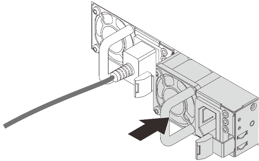
图 39. 安装热插拔电源模块
