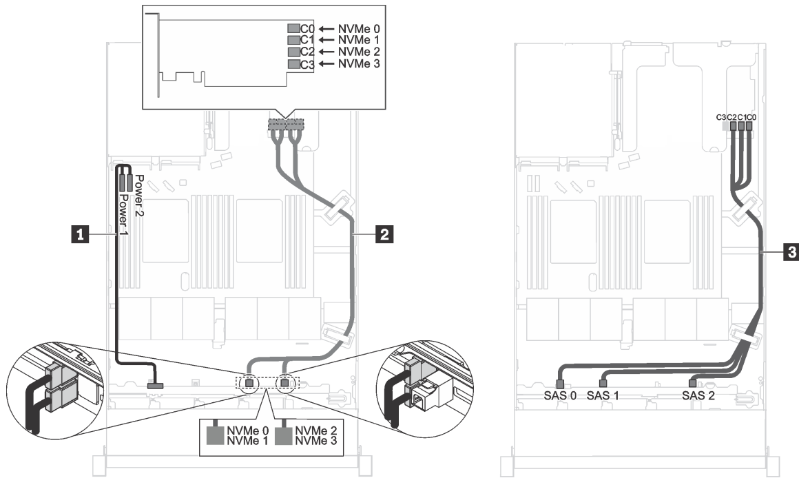
图 20. 配备六个 2.5 英寸 SAS/SATA 硬盘、四个 2.5 英寸 NVMe 硬盘、一个 16i RAID 适配器 (PCIe 插槽 1 中) 和一个 1610-4P NVMe 交换适配器 (PCIe 插槽 2 中) 的服务器型号的线缆布放
