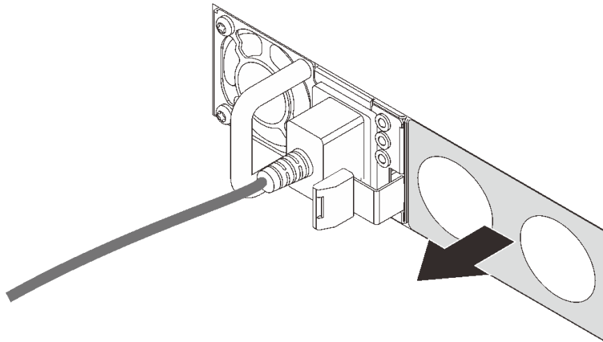
图 38. 卸下热插拔电源模块填充件
