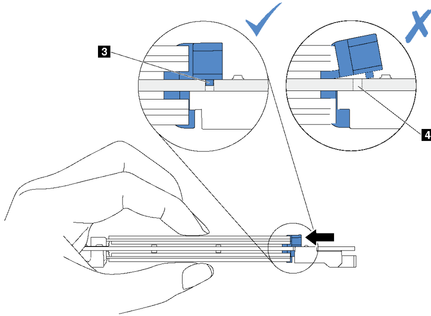
图 34. 关于滑动固定器的说明
