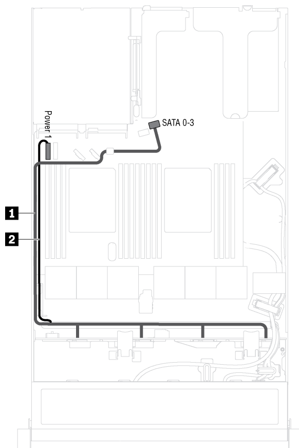
图 22. 配备四个 3.5 英寸易插拔硬盘的服务器型号的线缆布放
