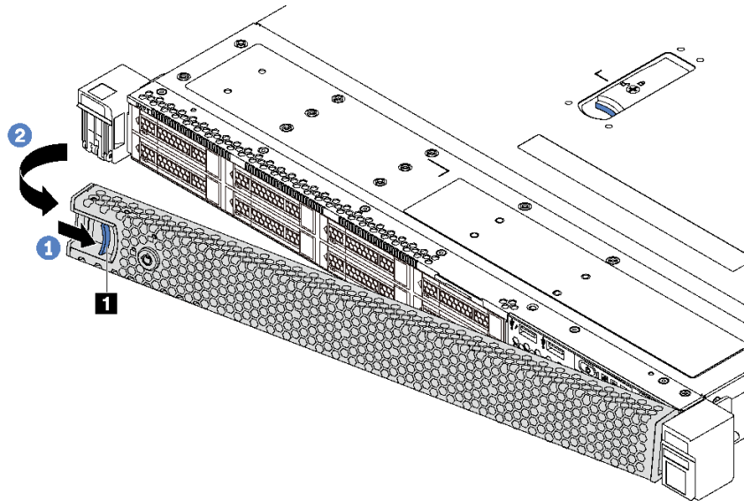
图 25. 卸下安全挡板
