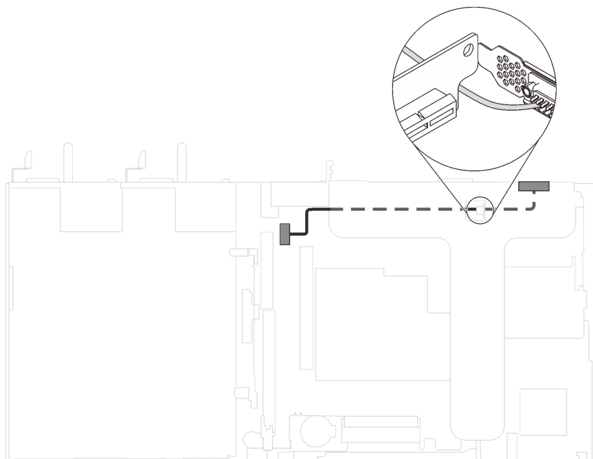
图 47. 安装在 PCIe 插槽 1 中的串口模块的线缆布放
