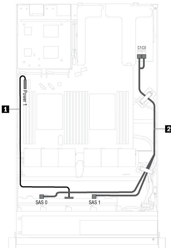
图 16. 配备八个 2.5 英寸热插拔硬盘的服务器型号的线缆布放
