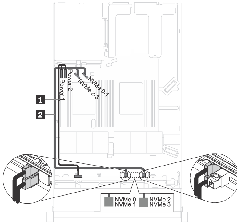
图 21. 配备四个 2.5 英寸 NVMe 硬盘且无 RAID 适配器的服务器型号的线缆布放
