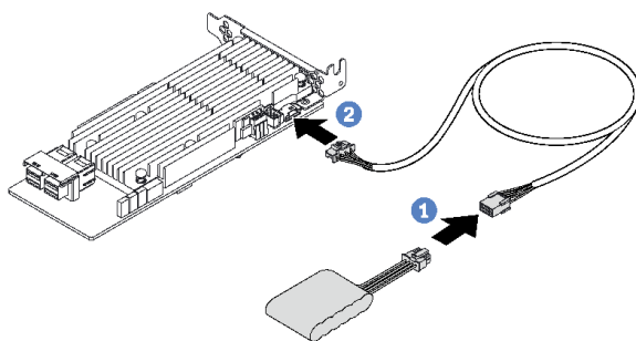
图 12. 将 RAID 超级电容器模块连接到 RAID 适配器
