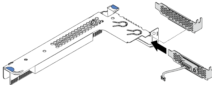
图 46. 安装串口模块
