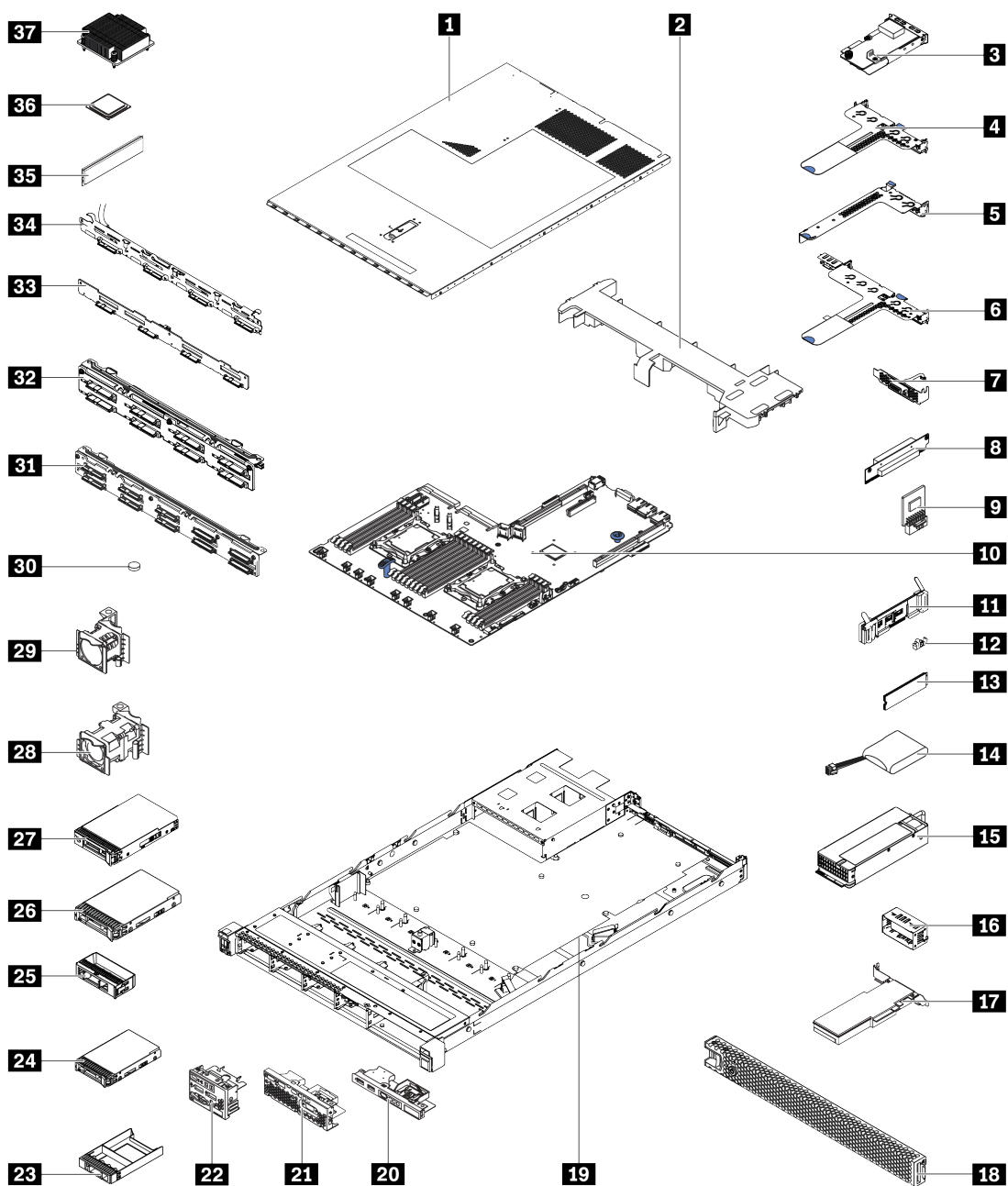
图 23. 服务器组件
