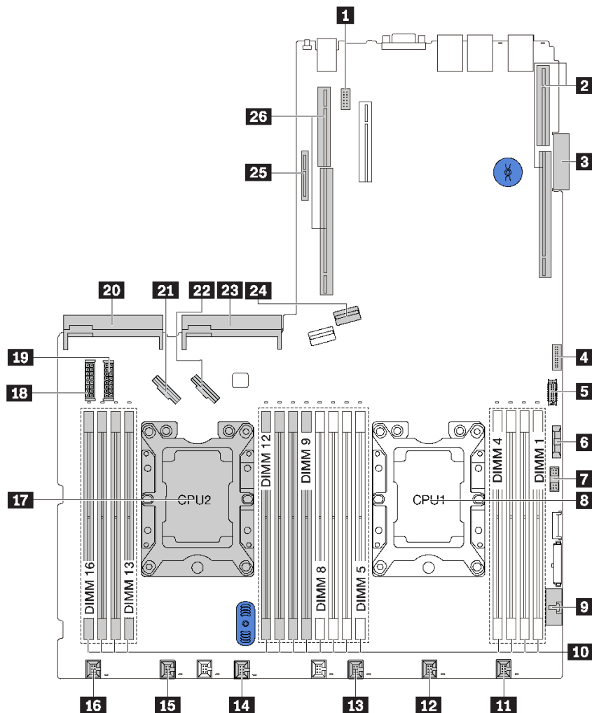
图 11. 主板组件
