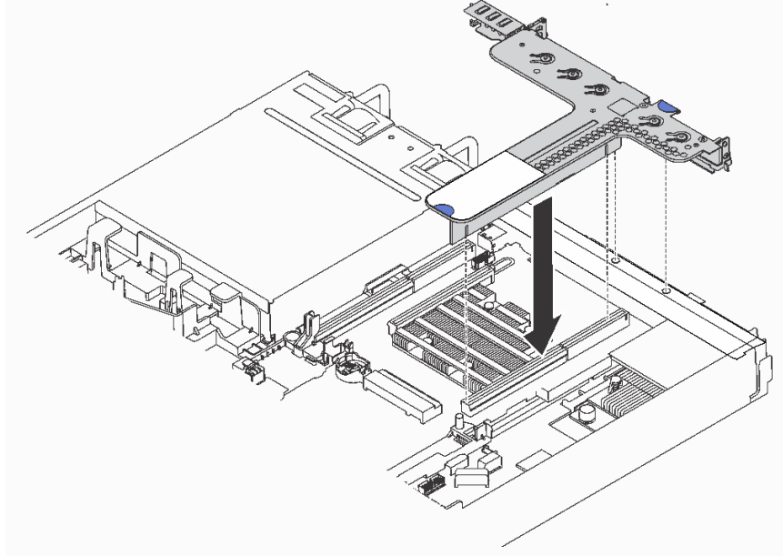
图 44. 安装转接卡组合件
