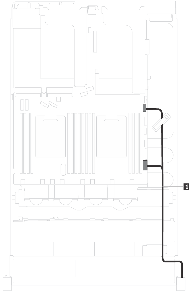
그림 18. 오른쪽 랙 래치의 앞면 입/출력 어셈블리에 대한 케이블 배선
