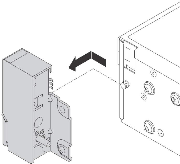
그림 39. 랙 래치 제거
