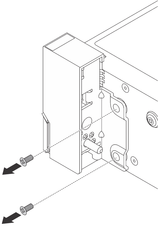
그림 38. 나사 제거
