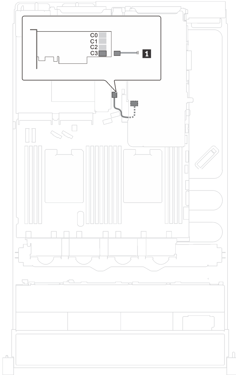
그림 97. 뒷면 핫 스왑 드라이브 어셈블리의 케이블 배선
