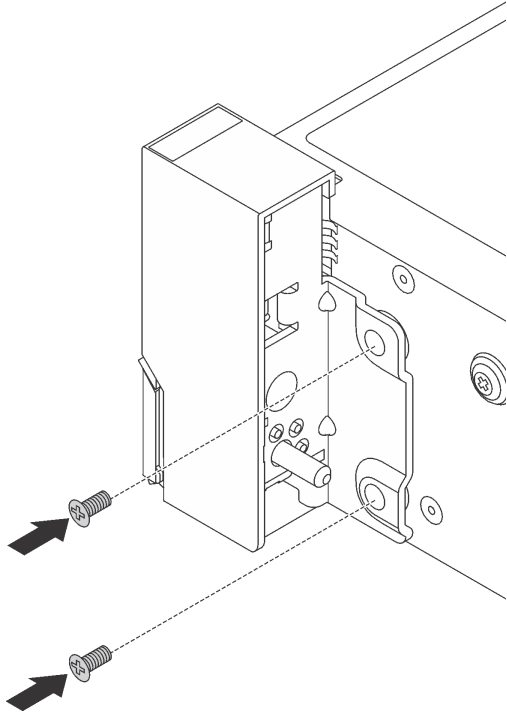
그림 41. 나사 설치
