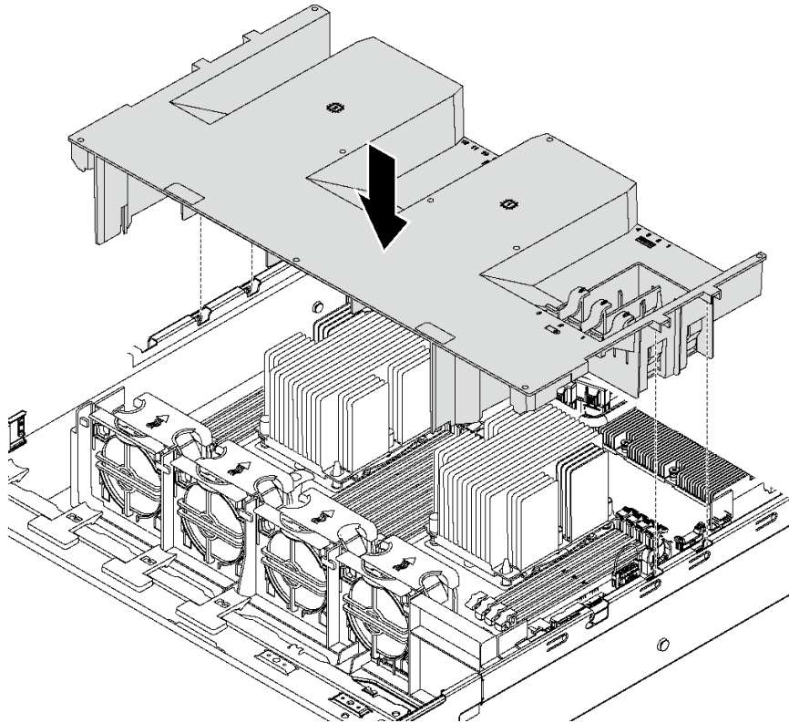
그림 51. 공기 조절 장치 설치
