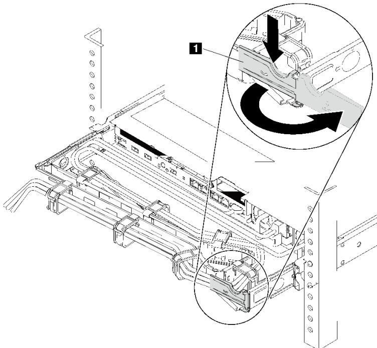
그림 115. CMA 조정
