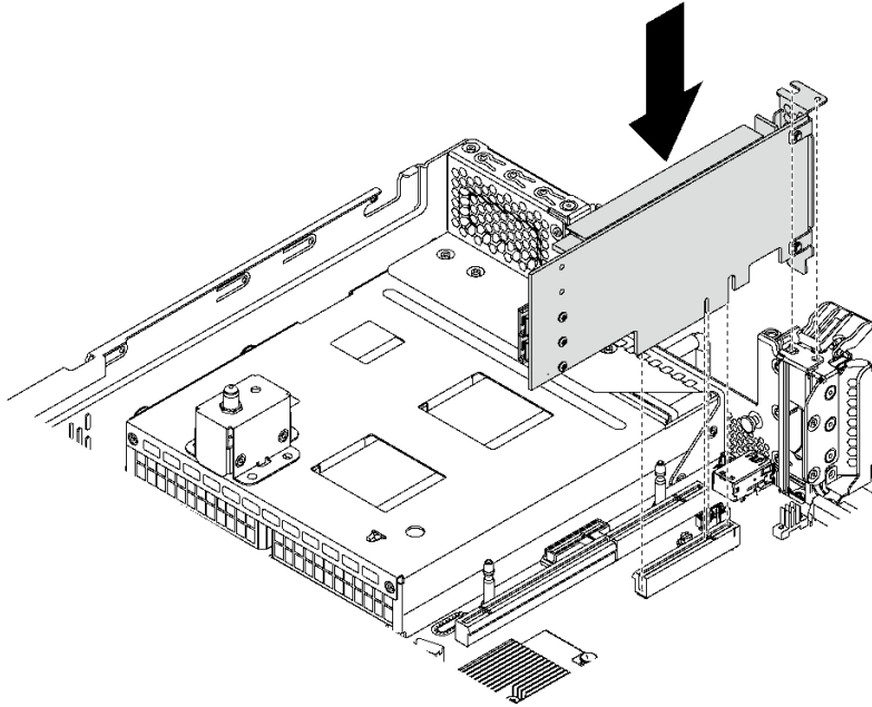
그림 94. 시스템 보드에 PCIe 어댑터 설치
