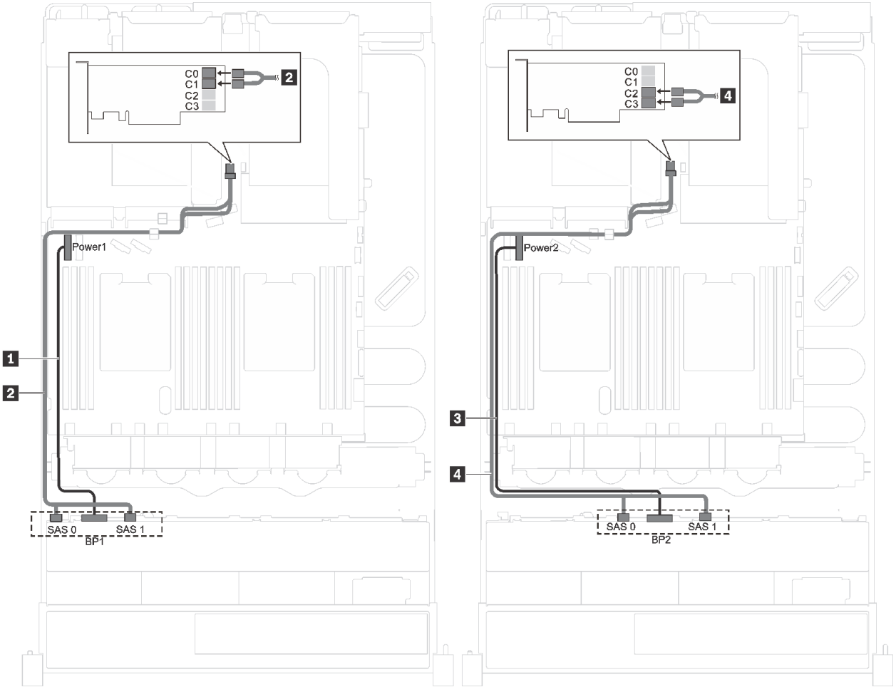
그림 22. 16개의 2.5인치 SAS/SATA 드라이브 및 1개의 16i RAID/HBA 어댑터가 있는 서버 모델의 케이블 배선
