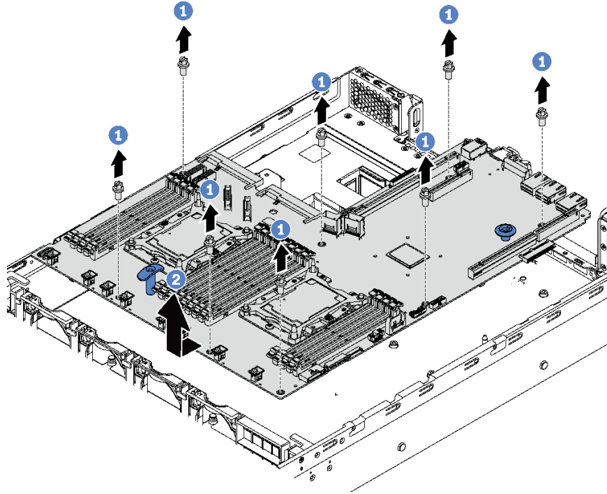
그림 128. 시스템 보드 제거
