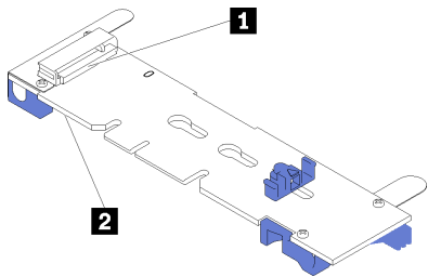
그림 106. M.2 드라이브 슬롯
