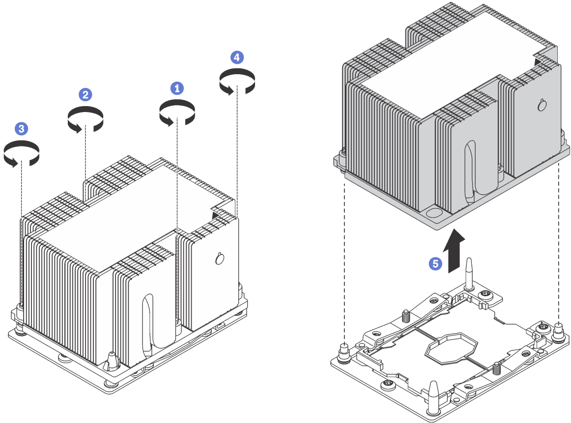
그림 120. PHM 제거
