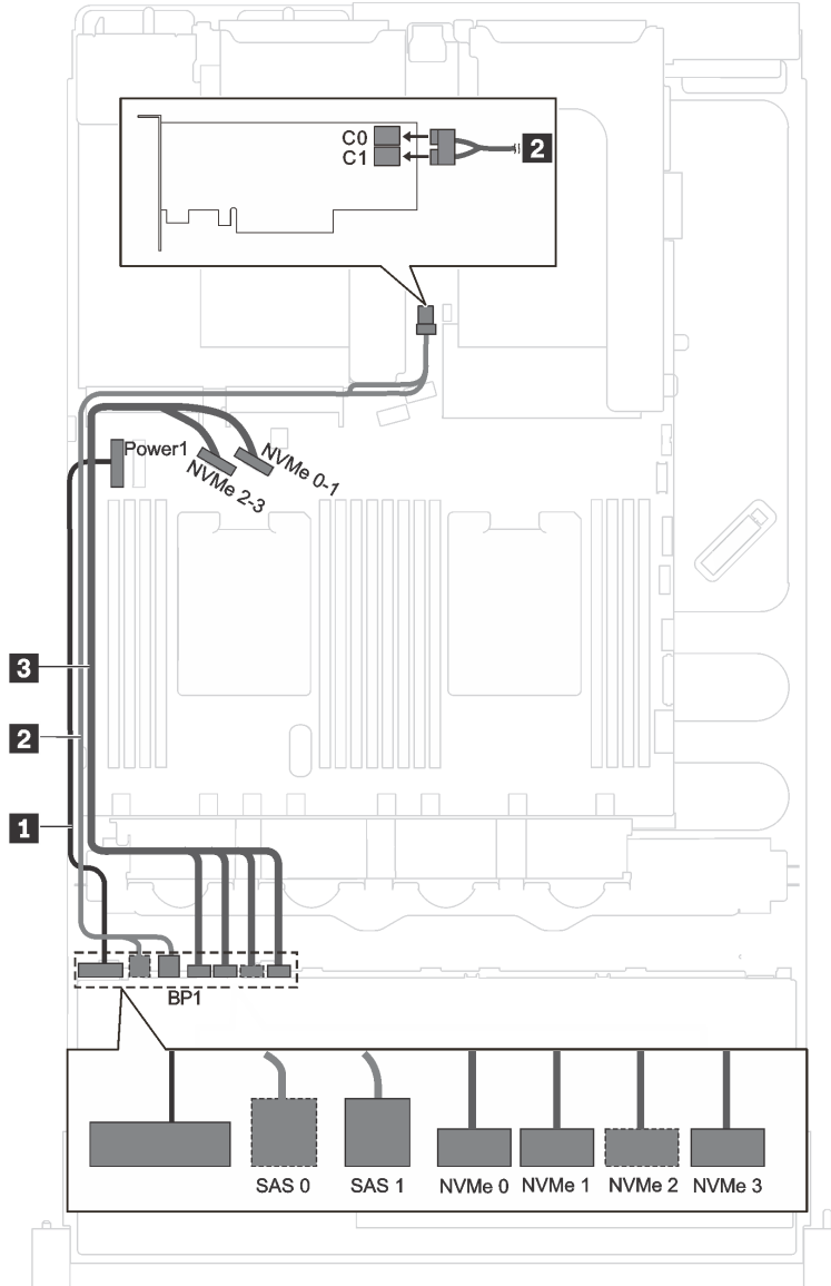
그림 20. 4개의 2.5인치 SAS/SATA 드라이브, 4개의 2.5인치 SAS/SATA/NVMe 드라이브, 1개의 8i SAS 어댑터 및 1개의 8i RAID/HBA 어댑터가 있는 서버 모델의 케이블 배선
