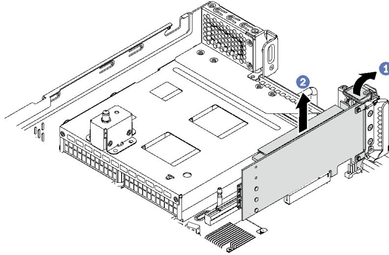
그림 91. 시스템 보드에서 PCIe 어댑터 제거
