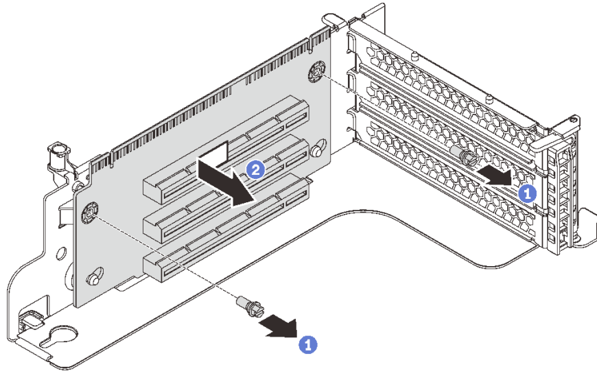
그림 84. 라이저 카드 제거
