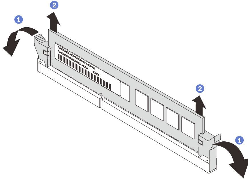
그림 77. 메모리 모듈 제거
