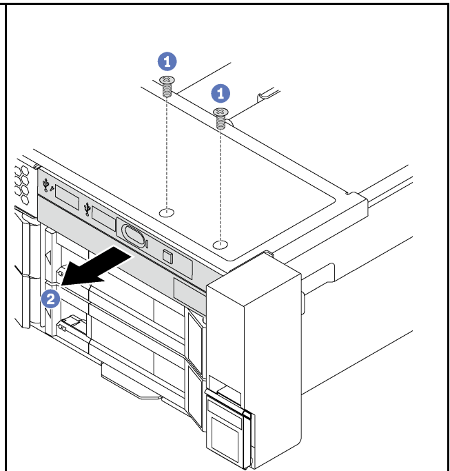
그림 57. 3.5인치 드라이브 베이이 있는 서버 모델
