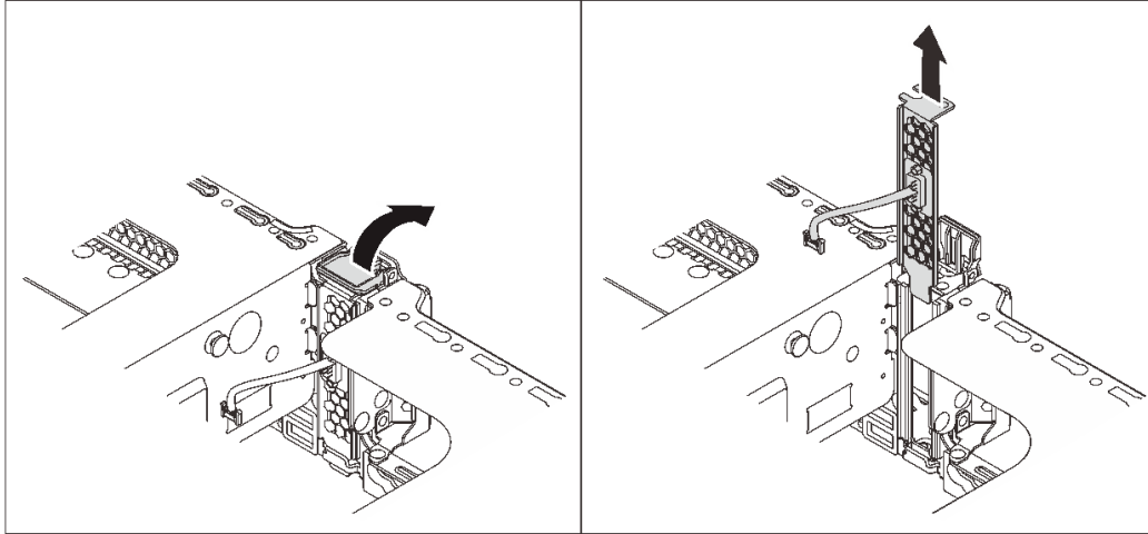
그림 100. 직렬 포트 모듈 제거
