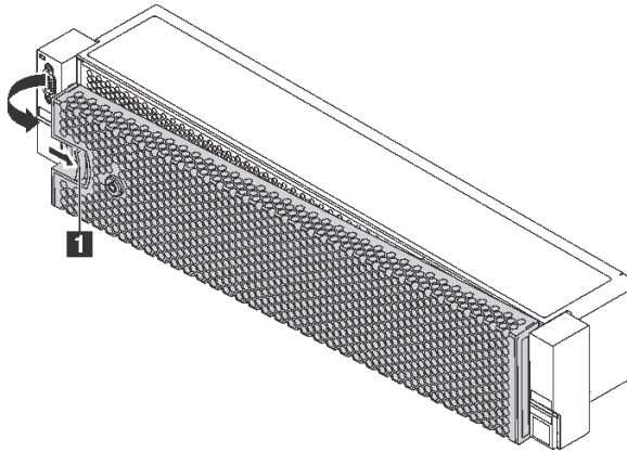
그림 31. 보안 베젤 제거
