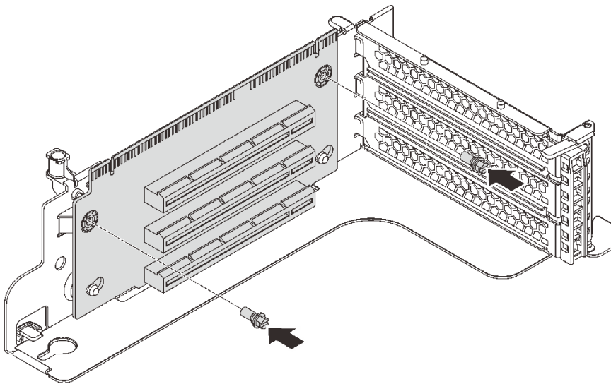
그림 86. 나사를 조여 라이저 카드 고정
