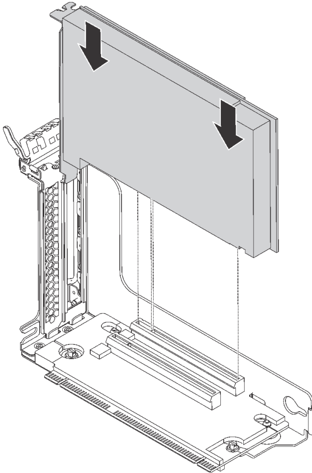
그림 92. PCIe 어댑터 설치
