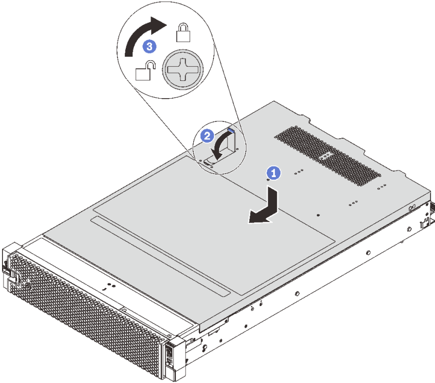
그림 46. 윗면 덮개 설치
