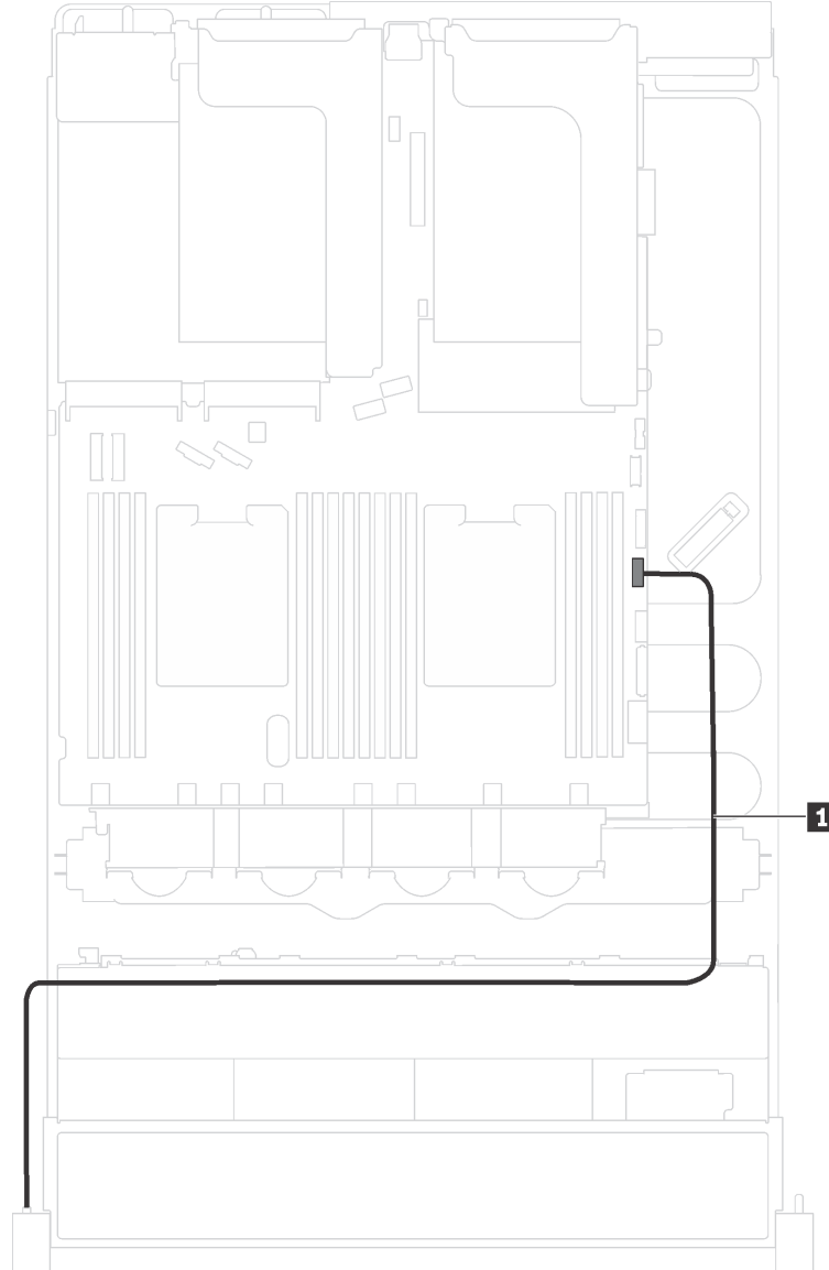
그림 16. VGA 커넥터 케이블 배선
