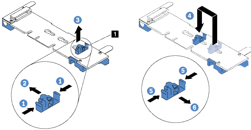
그림 105. M.2 고정장치 조정
