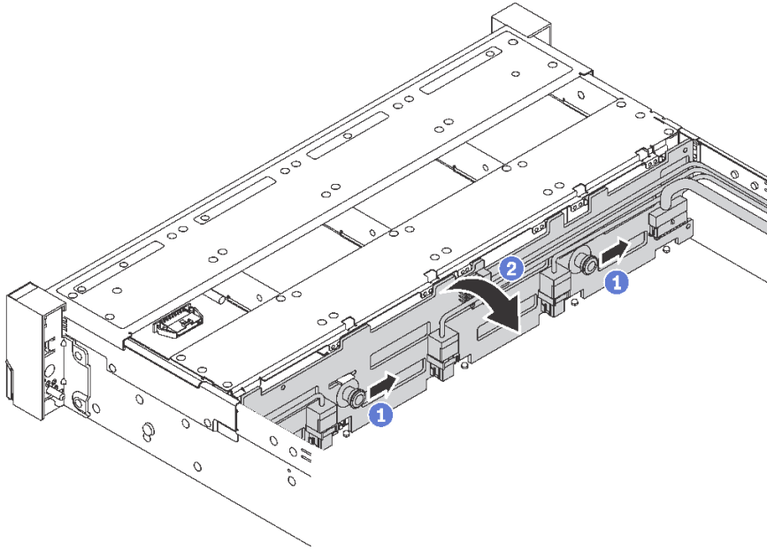
그림 73. 3.5인치 드라이브 백플레인 제거
