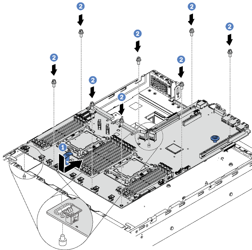
그림 129. 시스템 보드 설치
