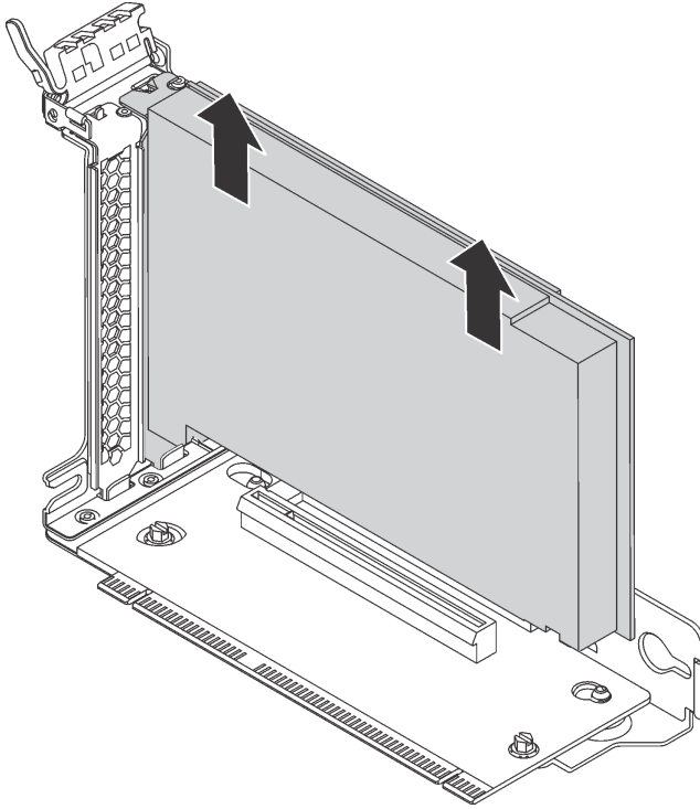
그림 90. 라이저 어셈블리에서 PCIe 어댑터 제거
