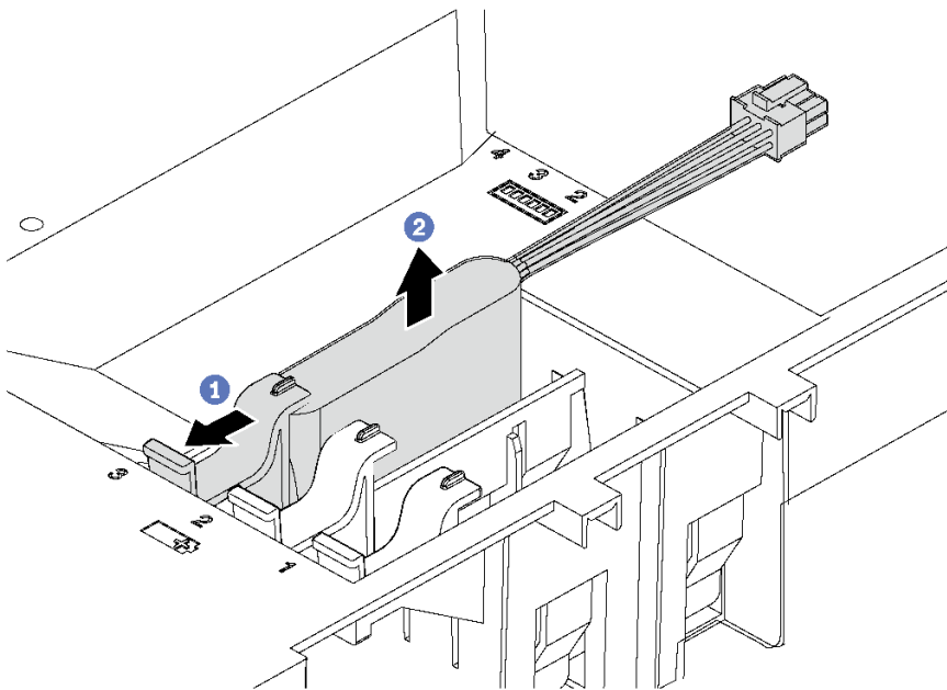
그림 47. RAID 슈퍼 캐패시터 모듈 제거
