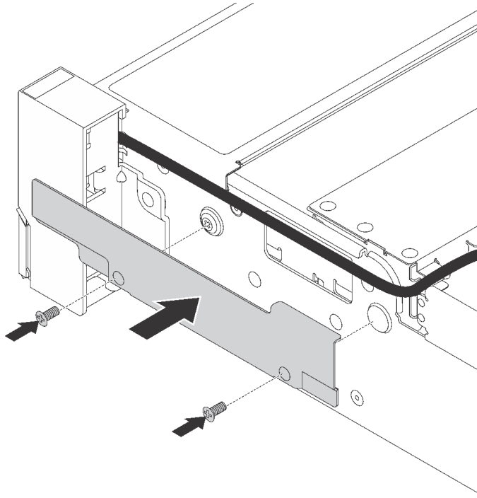
그림 42. 케이블 고정장치 설치
