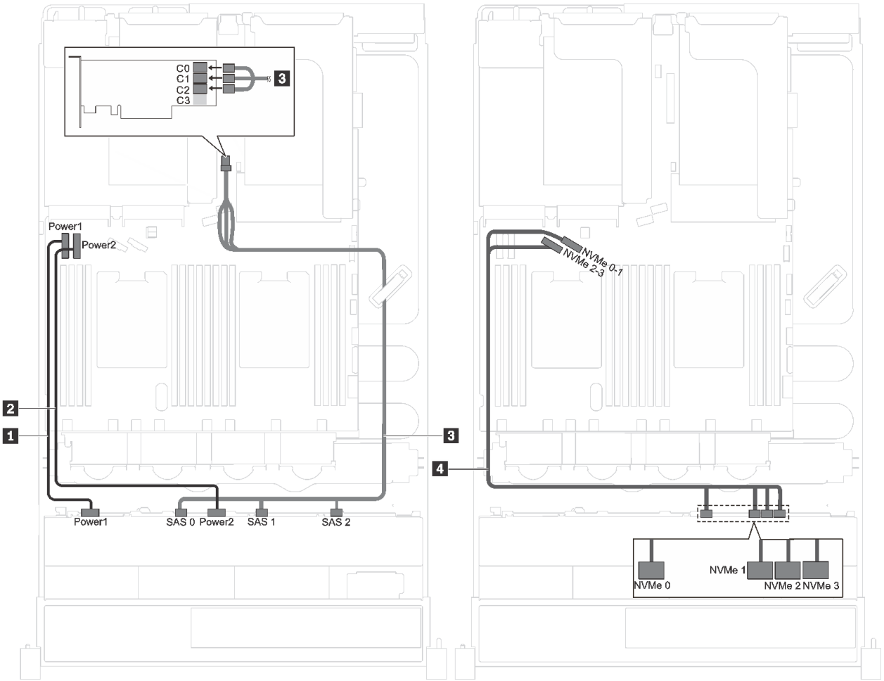
그림 28. 8개의 3.5인치 SAS/SATA 드라이브, 4개의 3.5인치 SAS/SATA/NVMe 드라이브 및 1개의 16i RAID/HBA 어댑터가 있는 서버 모델의 케이블 배선
