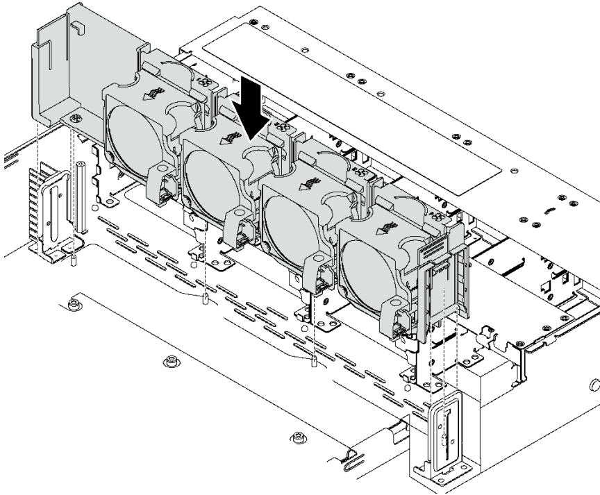
그림 55. 시스템 팬 케이스 설치
