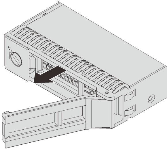
그림 69. 3.5인치 심플 스왑 드라이브 제거
