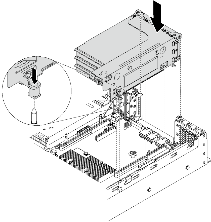
그림 87. 라이저 1 어셈블리 설치
