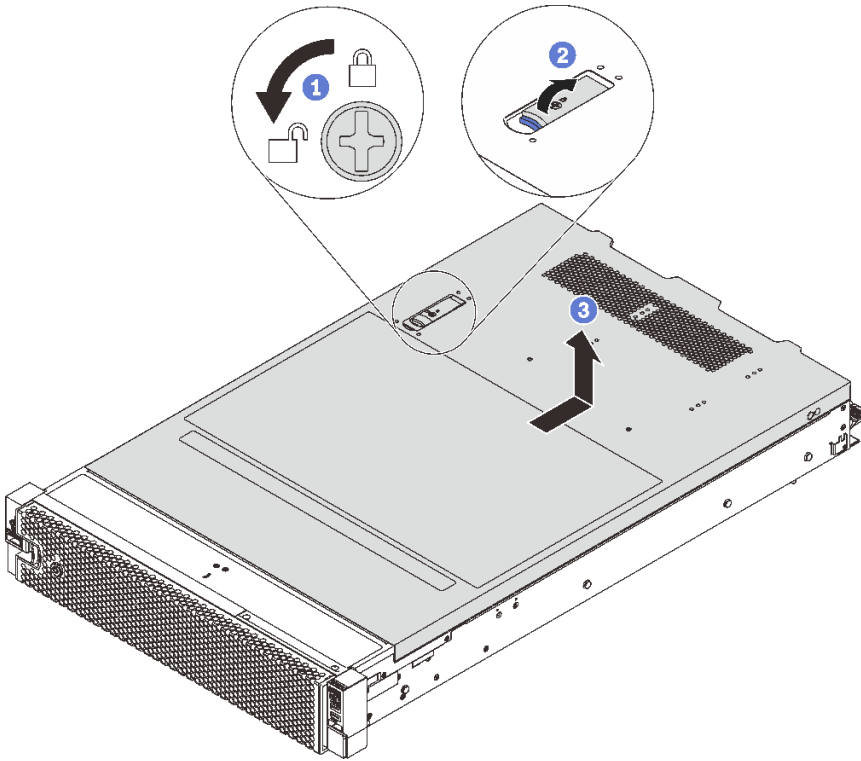
그림 45. 윗면 덮개 제거
