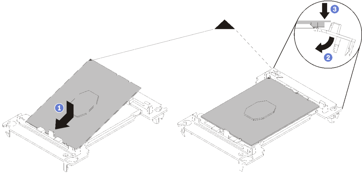
그림 123. 프로세서 고정장치 설치
