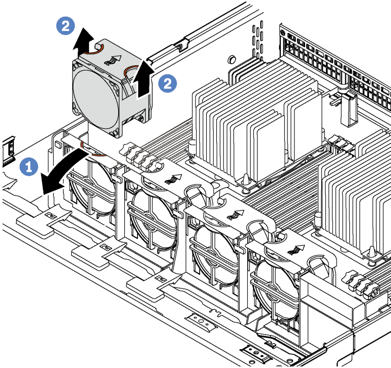
그림 52. 시스템 팬 제거
