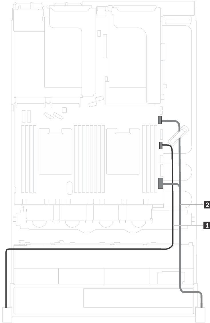
그림 43. 랙 래치에서 VGA 커넥터 및 전면 입/출력 어셈블리의 케이블 배선
