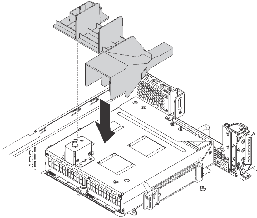
그림 110. M.2 드라이브 공기 조절 장치 설치
