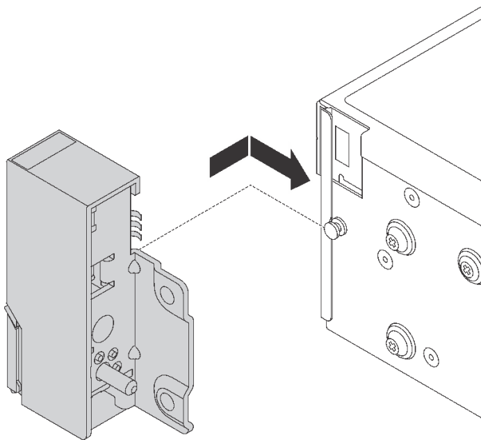
그림 40. 랙 래치 설치
