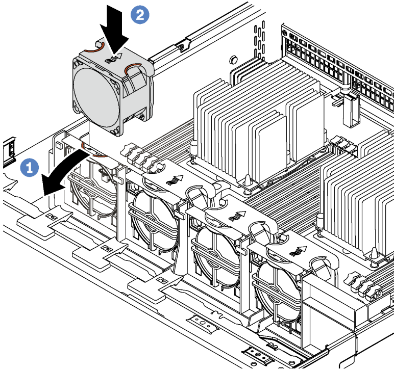
그림 53. 시스템 팬 설치
