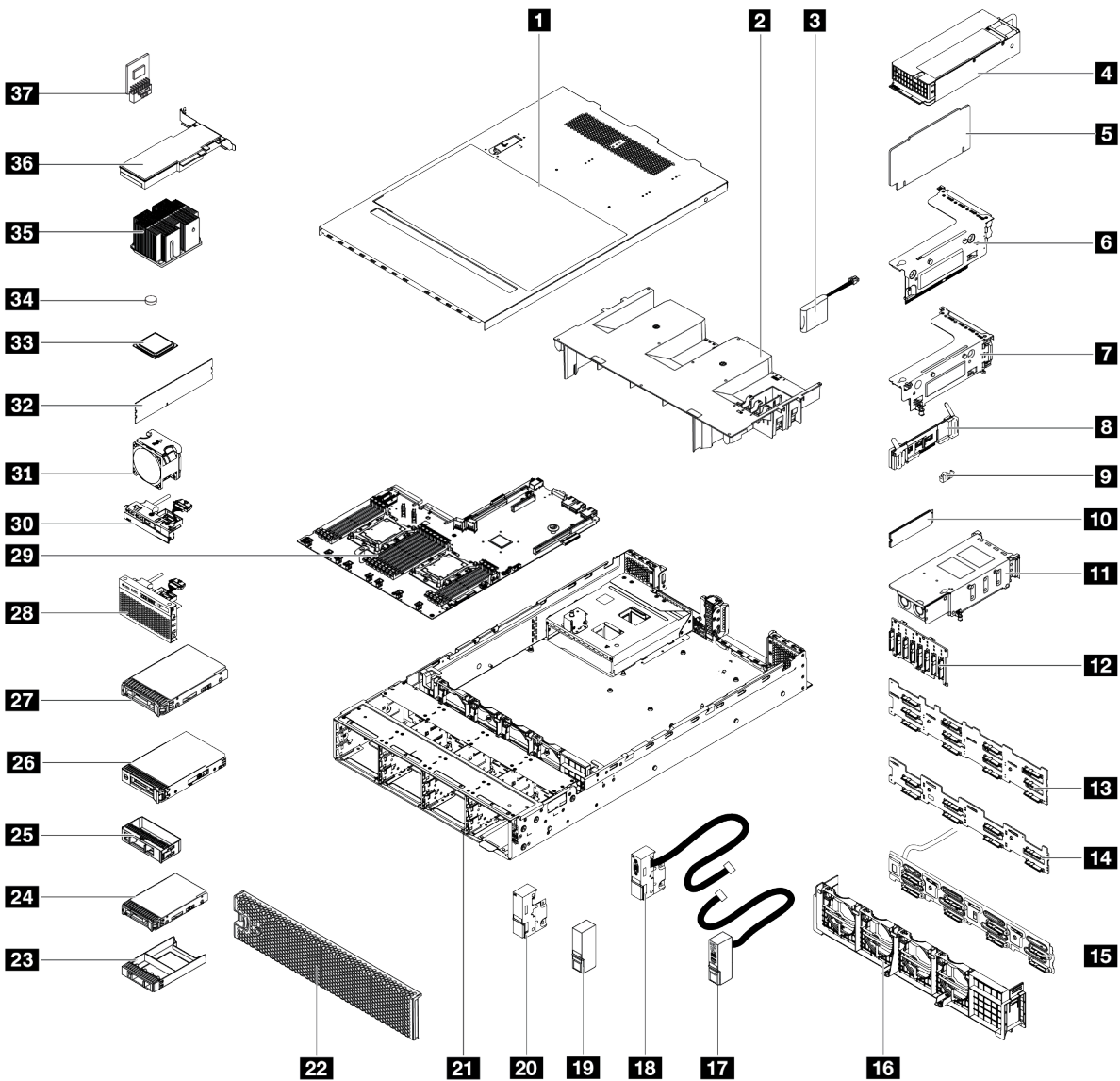
그림 29. 서버 구성 요소
