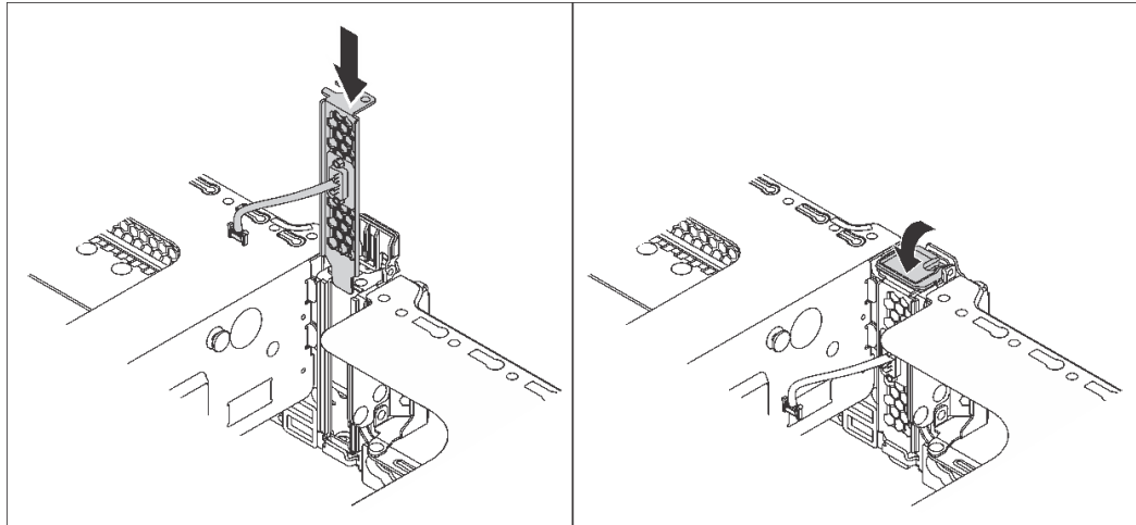
그림 101. 직렬 포트 모듈 설치
