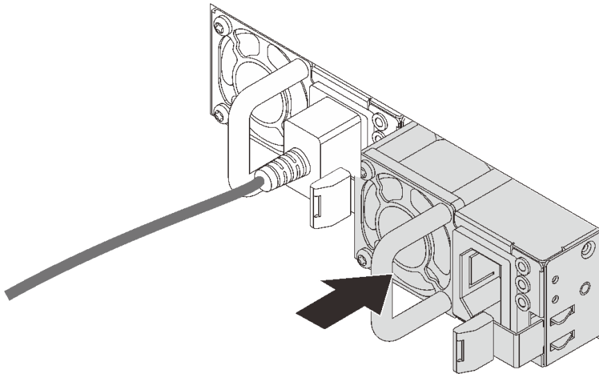
그림 117. 핫 스왑 전원 공급 장치 설치
