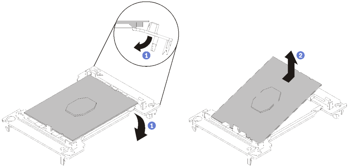
그림 122. 프로세서 고정장치 제거
