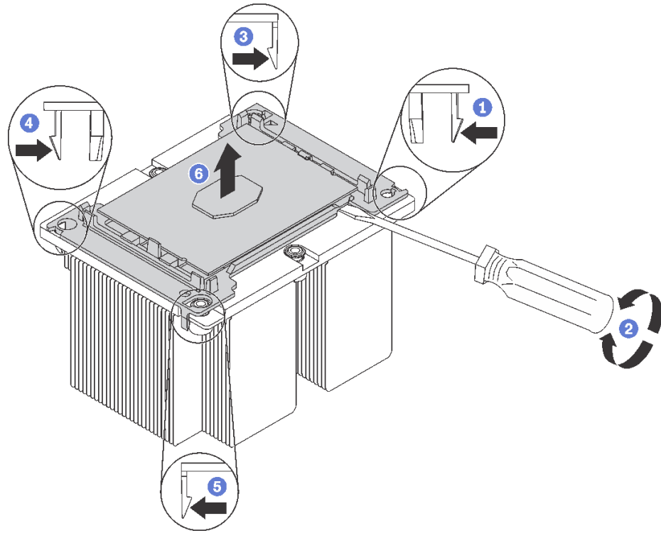
그림 121. 프로세서에서 방열판 분리
