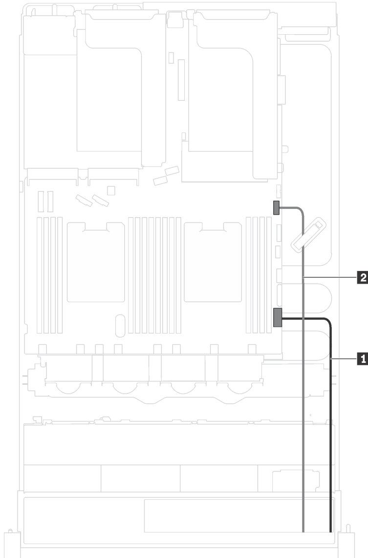
그림 17. 새시의 앞면 입/출력 어셈블리에 대한 케이블 배선
