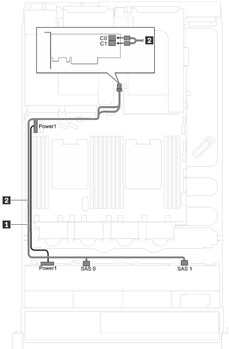
그림 24. 8개의 3.5인치 핫 스왑 드라이브 및 1개의 8i RAID/HBA 어댑터가 있는 서버 모델의 케이블 배선
