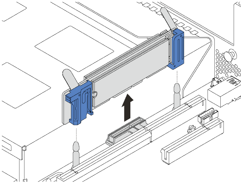
그림 103. M.2 백플레인 제거
