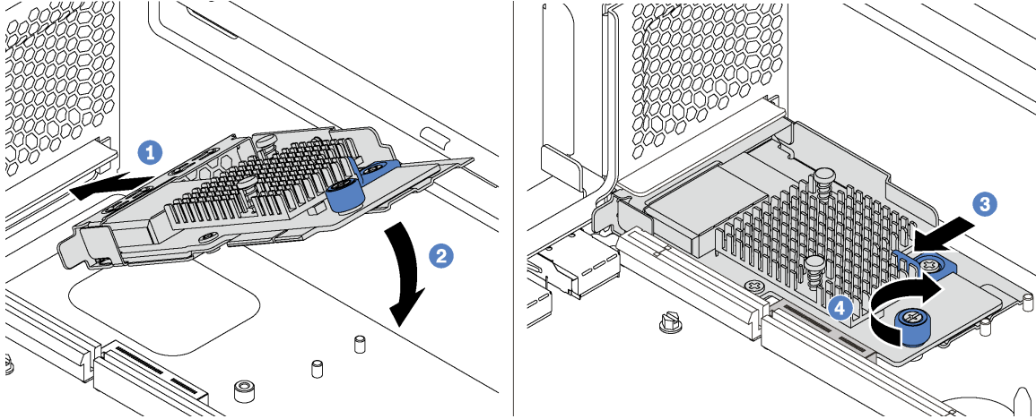
그림 99. LOM 어댑터 설치
