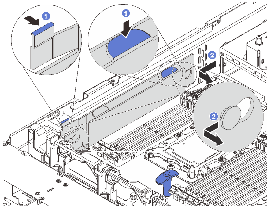
그림 127. 케이블 홀더 제거
