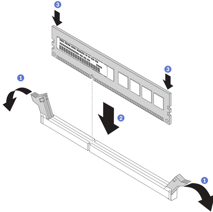
그림 78. 메모리 모듈 설치
