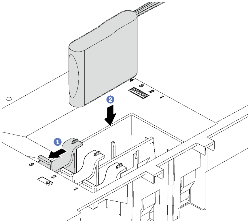
그림 48. RAID 슈퍼 캐패시터 모듈 설치
