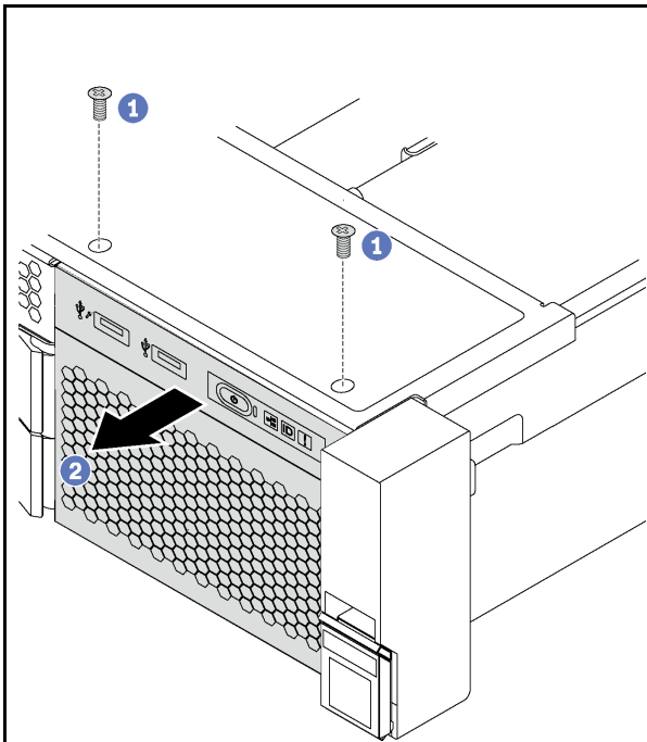
그림 56. 2.5인치 드라이브 베이이 있는 서버 모델
