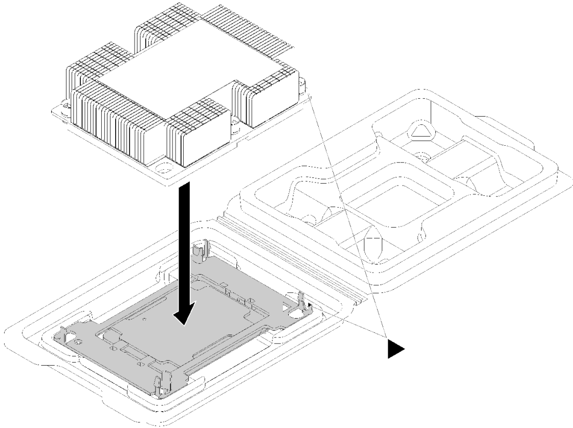
그림 125. 운송 트레이 내부의 PHM 조립
