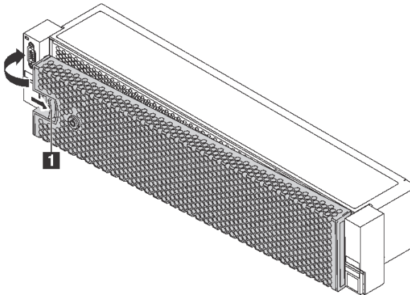
그림 33. 보안 베젤 설치
