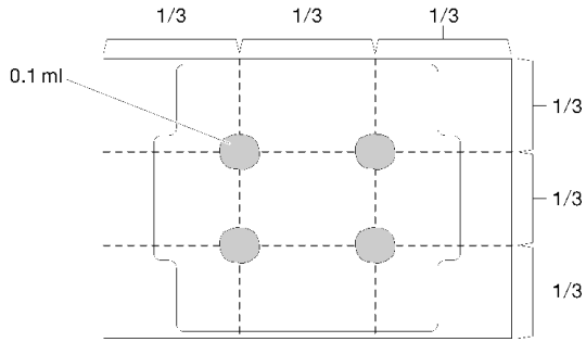
그림 124. 열전도 그리스 도포
