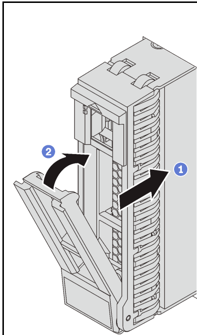
그림 66. 2.5인치 핫 스왑 드라이브 설치
