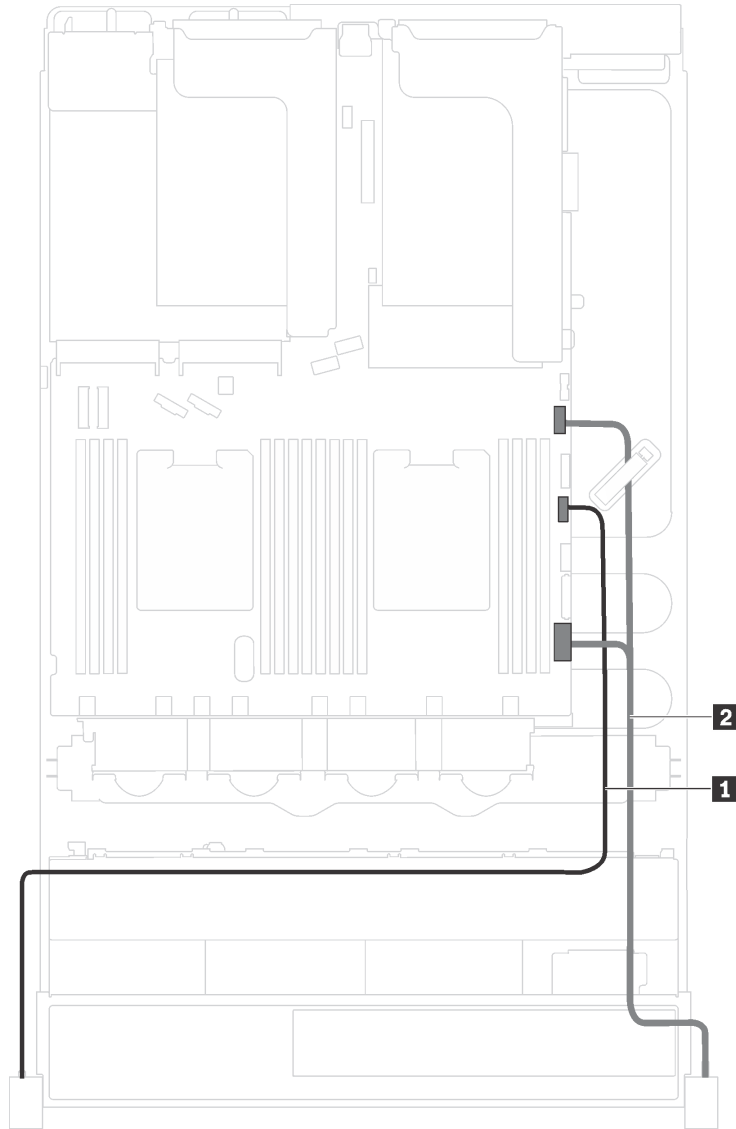
그림 36. 랙 래치에서 VGA 커넥터 및 전면 입/출력 어셈블리의 케이블 배선
