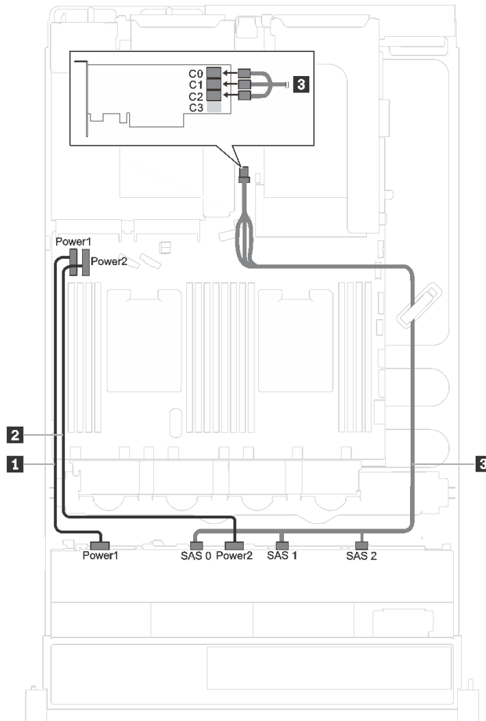
그림 26. 12개의 3.5인치 SAS/SATA 드라이브 및 1개의 16i RAID/HBA 어댑터가 있는 서버 모델의 케이블 배선
