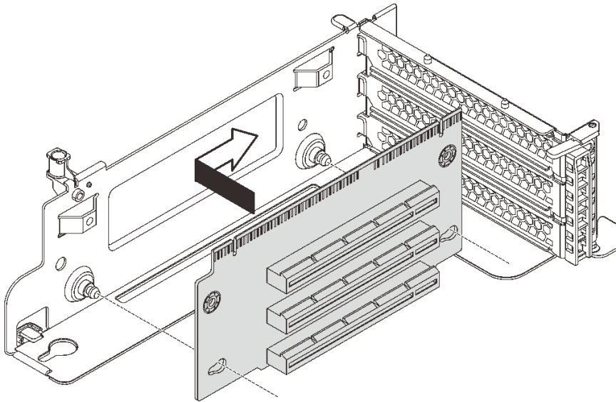
그림 85. 라이저 카드 설치
