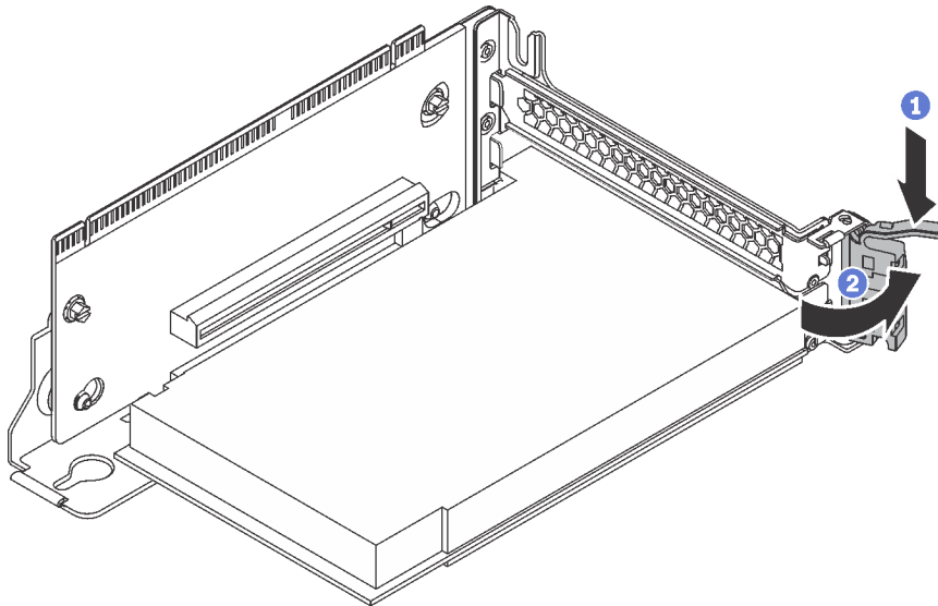
그림 89. PCIe 어댑터 고정 래치 열기
