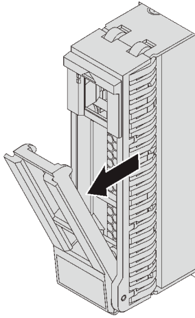
그림 62. 2.5인치 핫 스왑 드라이브 제거
