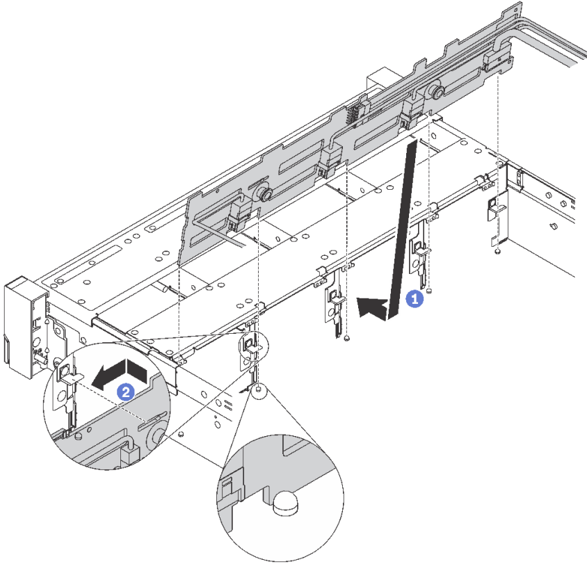
그림 74. 3.5인치 드라이브 백플레인 설치
