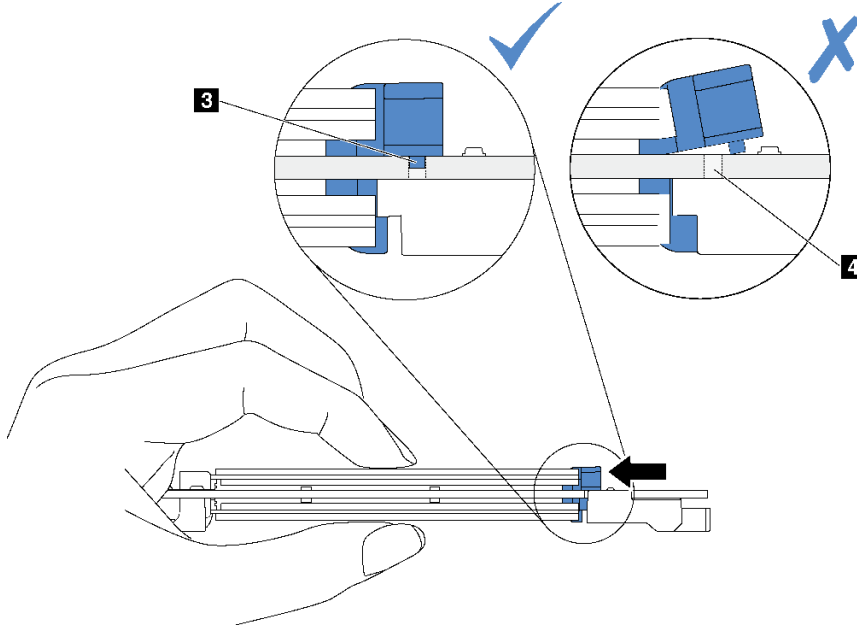
그림 108. 고정장치를 밀는 방법
