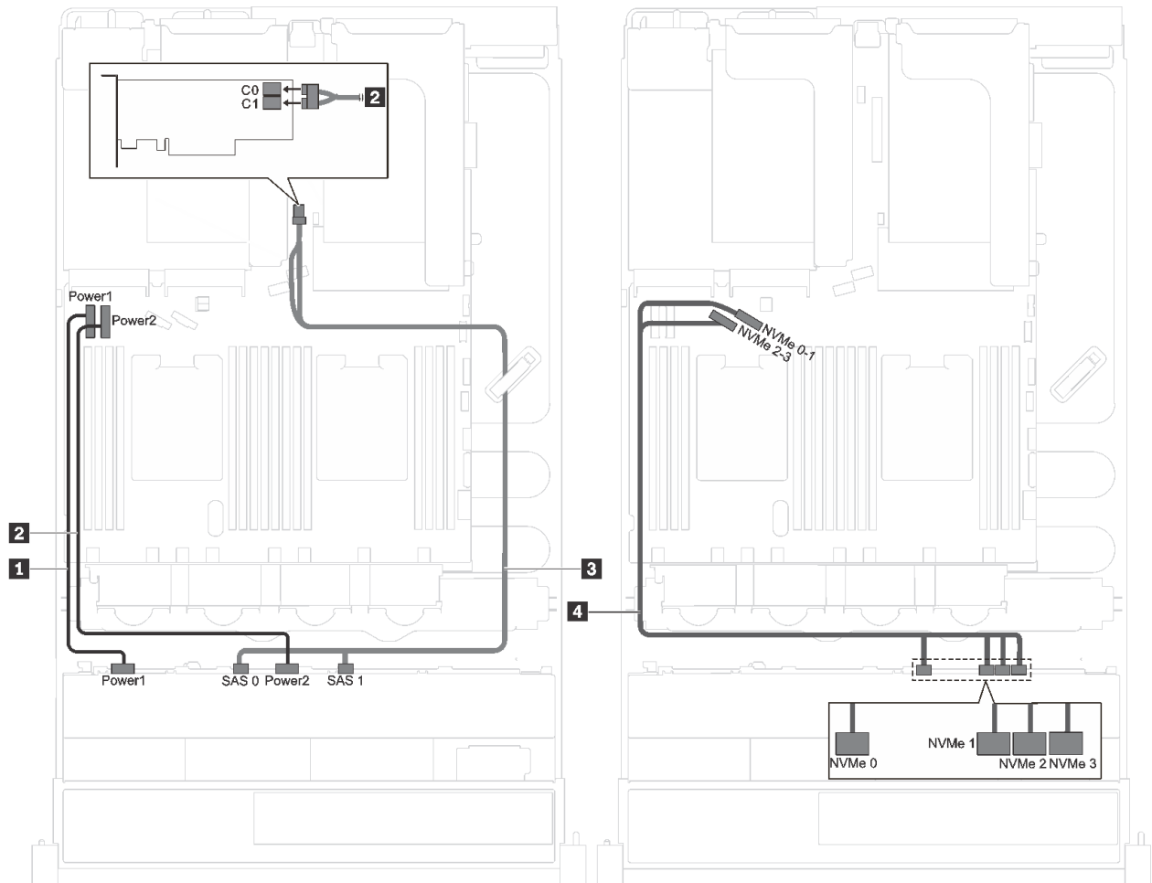
그림 27. 8개의 3.5인치 SAS/SATA 드라이브, 4개의 3.5인치 NVMe 드라이브 및 1개의 8i RAID/HBA 어댑터가 있는 서버 모델의 케이블 배선
