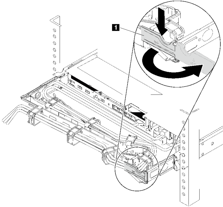
그림 112. CMA 조정
