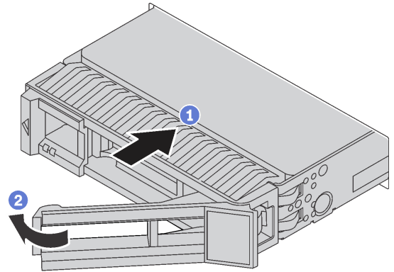
그림 67. 3.5인치 핫 스왑 드라이브 설치
