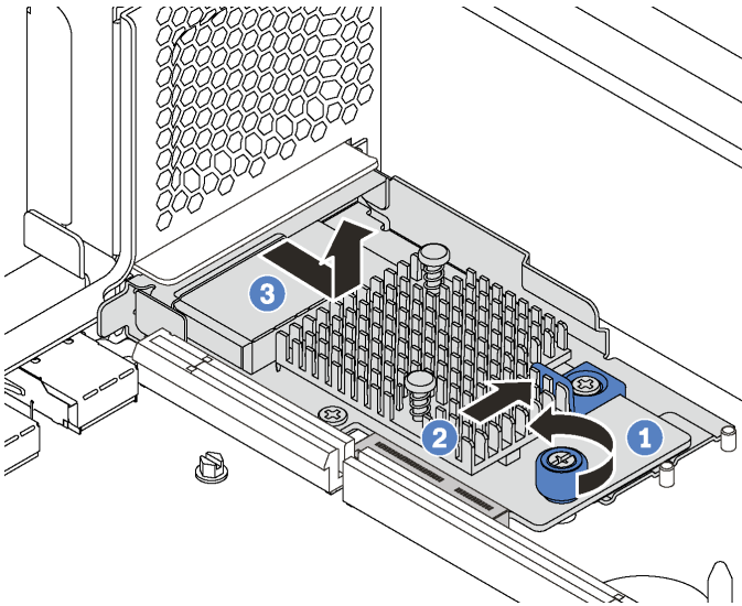
그림 98. LOM 어댑터 제거
