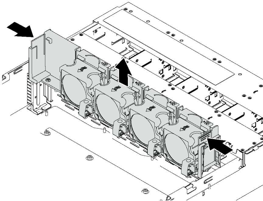
그림 54. 시스템 팬 케이스 제거
