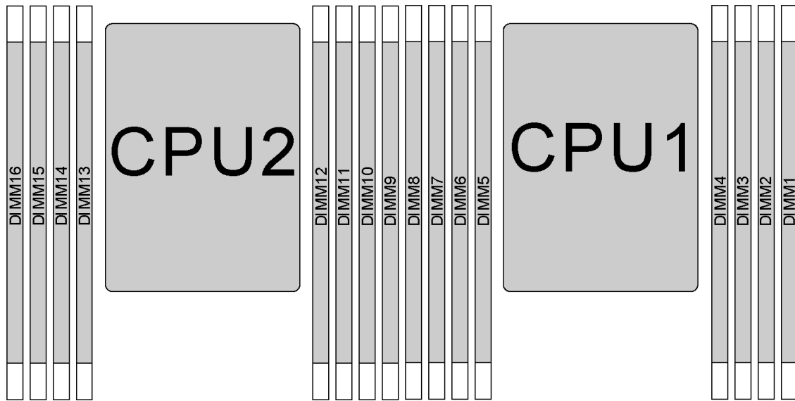
그림 79. DIMM 위치
