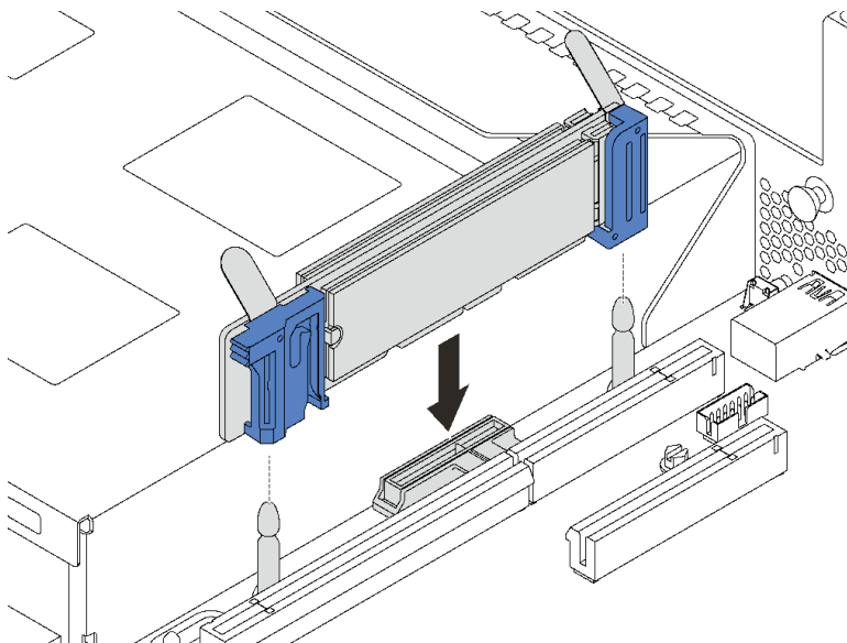
그림 109. M.2 백플레인 설치
