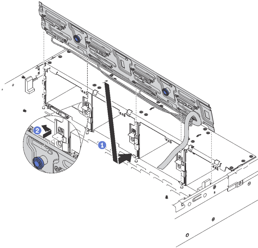
그림 76. 3.5인치 심플 스왑 드라이브 백플레이트 어셈블리 설치
