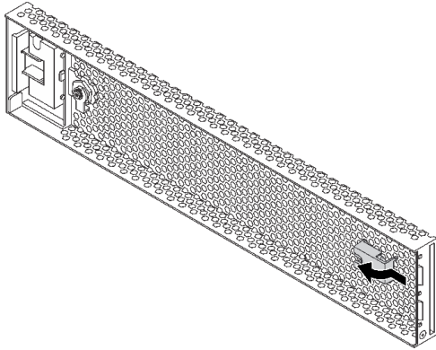
그림 32. 키 제거
