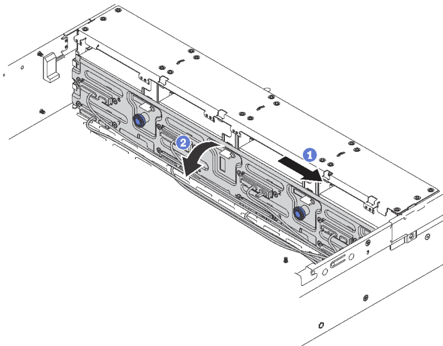
그림 75. 3.5인치 심플 스왑 드라이브 백플레이트 어셈블리 제거
