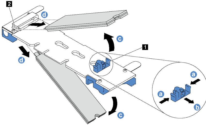
그림 104. M.2 드라이브 제거
