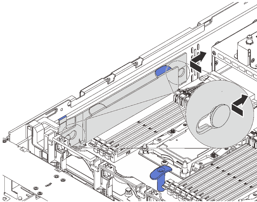
그림 130. 케이블 홀더 설치
