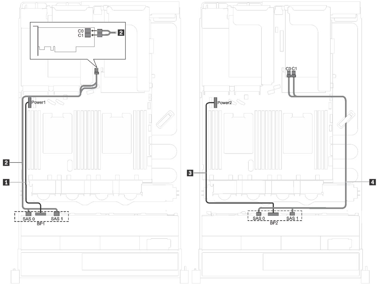
그림 21. 16개의 2.5인치 SAS/SATA 드라이브 및 2개의 8i RAID/HBA 어댑터가 있는 서버 모델의 케이블 배선
