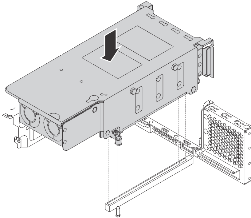
그림 96. 뒷면 핫 스왑 드라이브 어셈블리 설치
