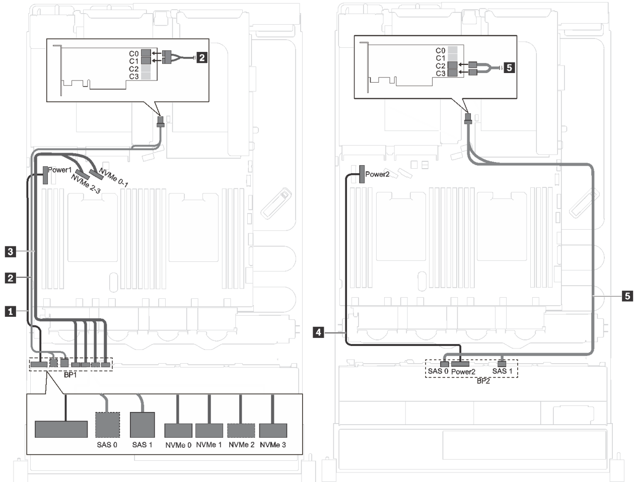
그림 23. 12개의 2.5인치 SAS/SATA 드라이브, 4개의 2.5인치 SAS/SATA/NVMe 드라이브 및 1개의 16i RAID/HBA 어댑터가 있는 서버 모델의 케이블 배선
