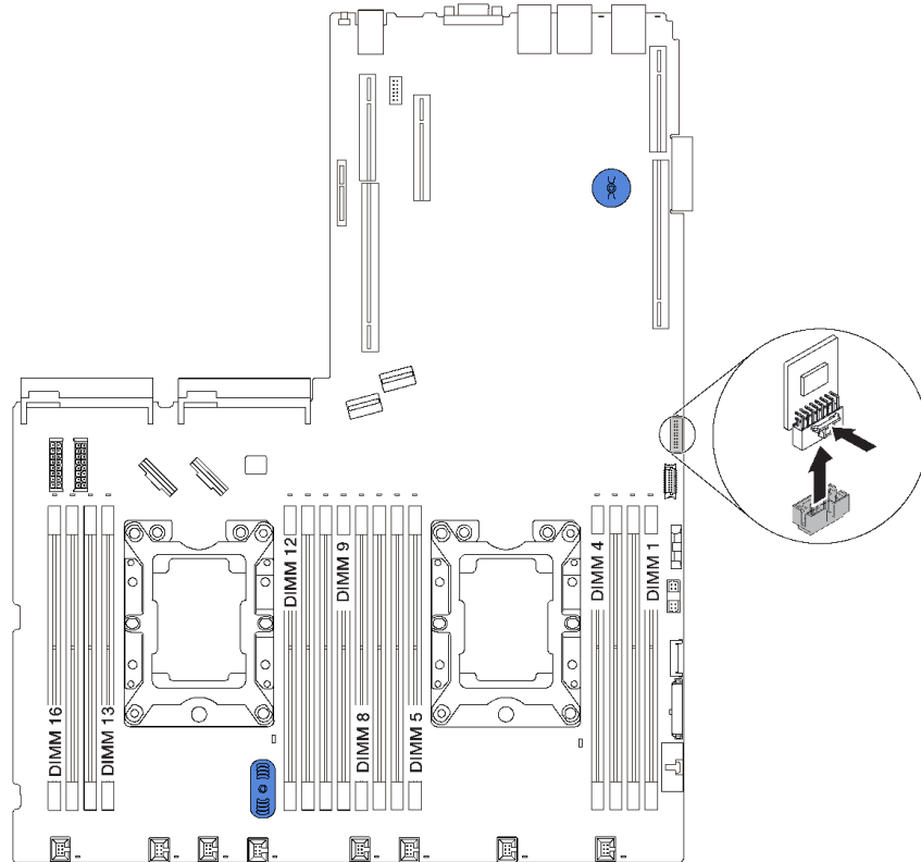
그림 118. TCM/TPM 어댑터 제거
