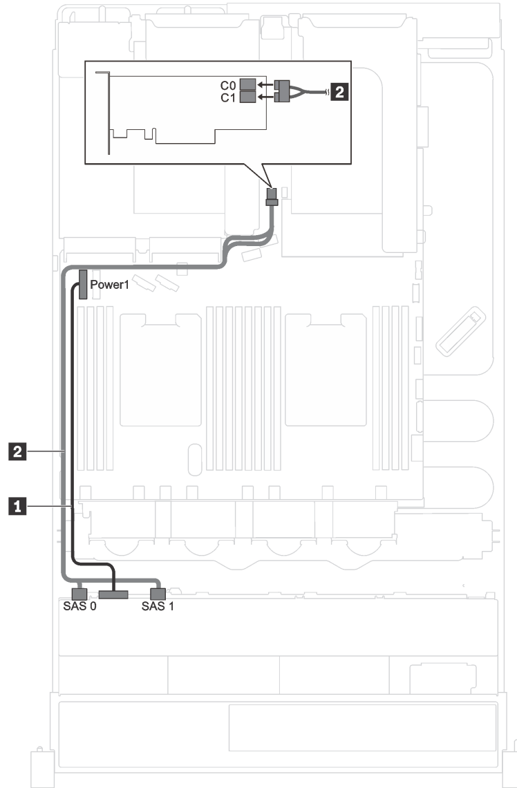
그림 19. 2.5인치 SAS/SATA 드라이브 8개 및 8i RAID/HBA 어댑터 1개가 지원되는 서버 모델의 케이블 배선
