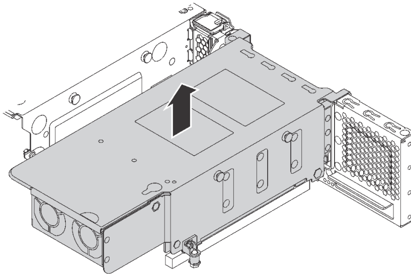
그림 95. 뒷면 핫 스왑 드라이브 어셈블리 제거
