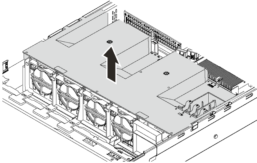
그림 50. 공기 조절 장치 제거
