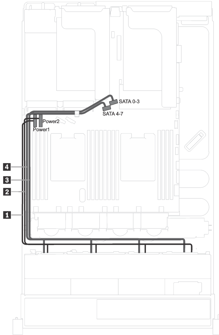
그림 25. 8개 3.5인치 심플 스왑 드라이브가 지원되는 서버 모델의 케이블 배선
