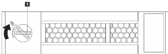
그림 68. 3.5인치 심플 스왑 드라이브의 손잡이 열기
