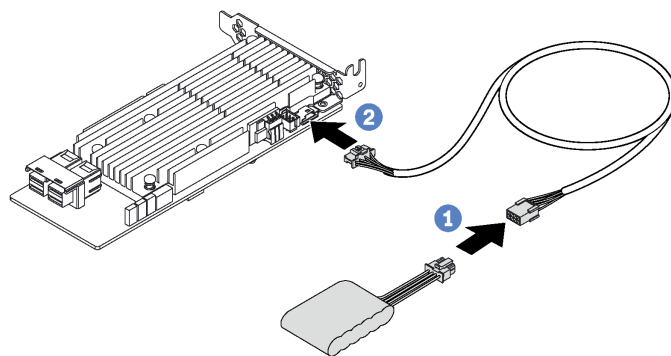
그림 49. RAID 슈퍼 캐패시터 모듈과 RAID 어댑터의 연결
