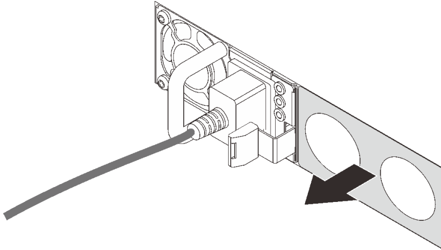
그림 116. 핫 스왑 전원 공급 장치 필터 제거
