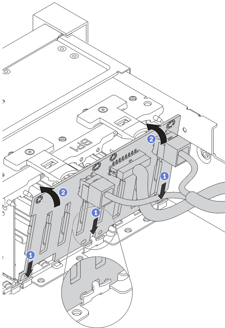
그림 72. 2.5인치 드라이브 백플레인 설치
