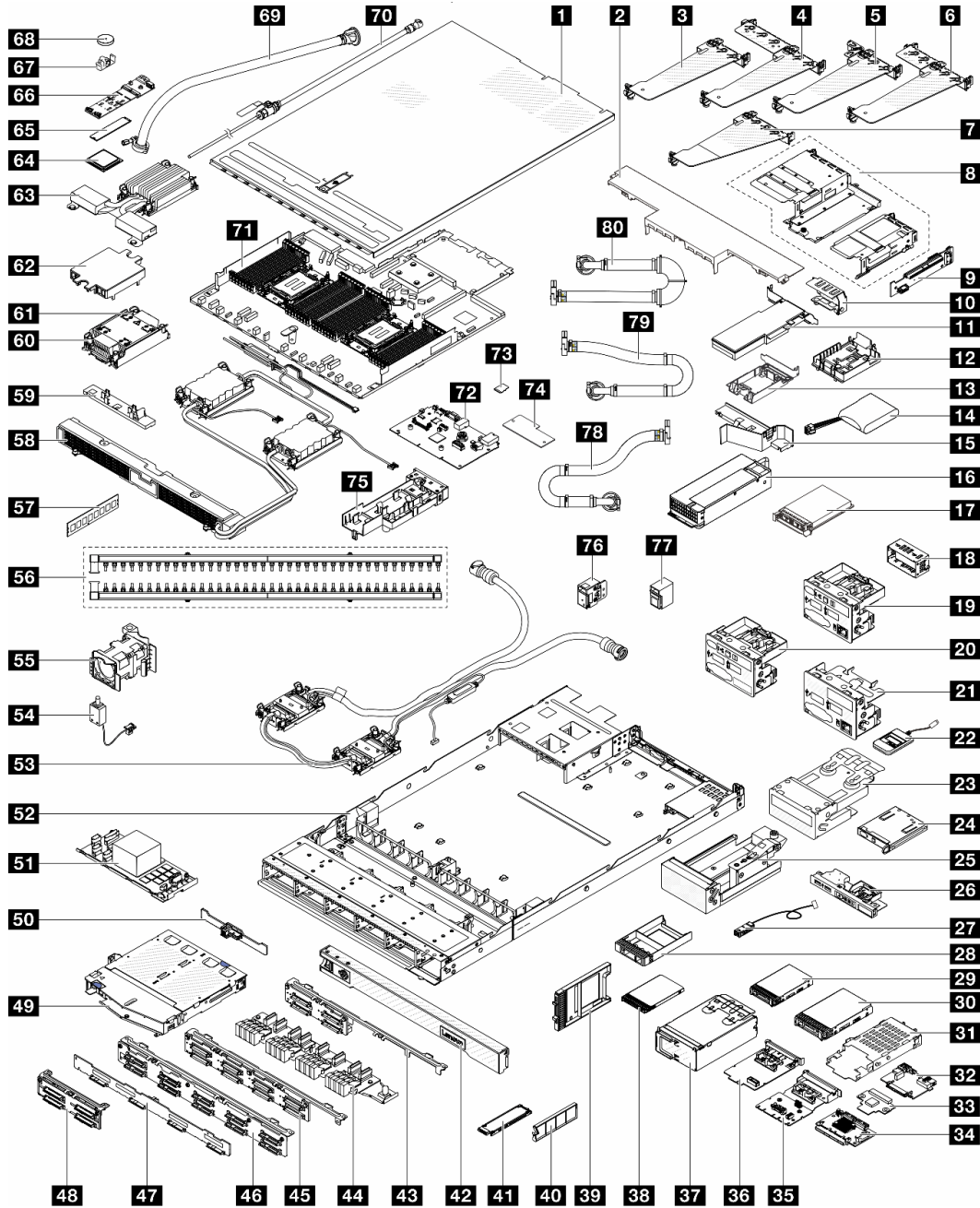
그림 26. 서버 구성 요소
