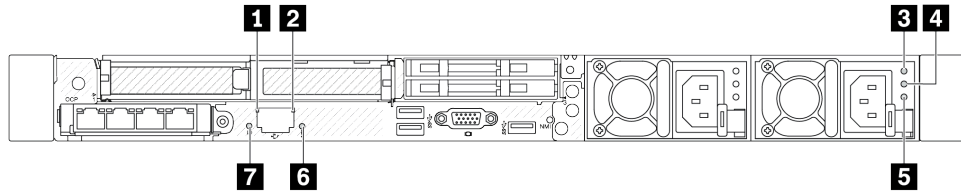
그림 22. 뒷면 LED 개요
