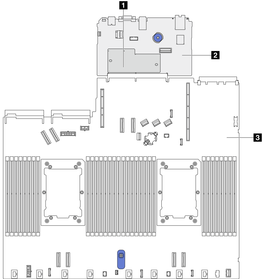
Рис. 14. Компоновка блока материнской платы
