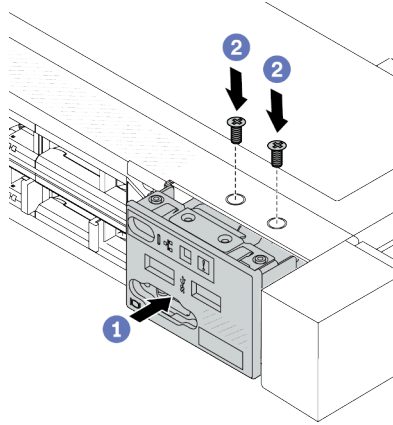
Рис. 76. Установка переднего модуля ввода-вывода в 2,5-дюймовую раму
