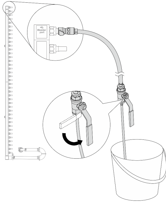
Рис. 138. Открытие клапана отводной трубки
