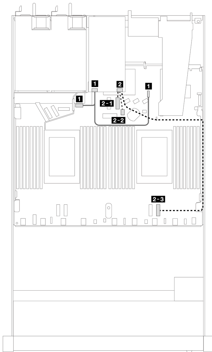
Рис. 342. Прокладка кабелей для дисков толщиной 7 мм
