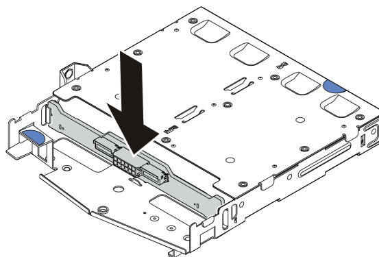
Рис. 225. Установка задней объединительной панели
