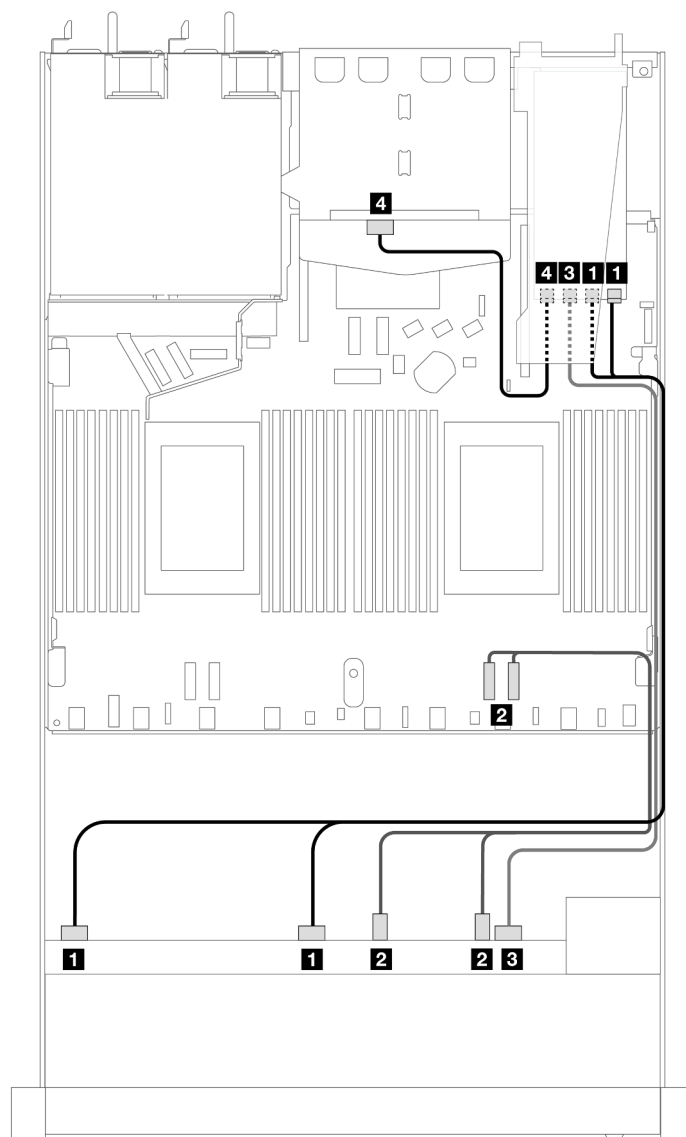
Рис. 458. Прокладка кабелей для шести передних дисков SAS/SATA, четырех отсеков для передних дисков AnyBay и адаптера RAID 16i SFF (Gen 3) с двумя установленными задними 2,5-дюймовыми дисками SAS/SATA
