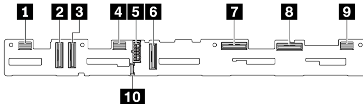
Рис. 304. Объединительная панель с 10 отсеками для 2,5-дюймовых дисков AnyBay
