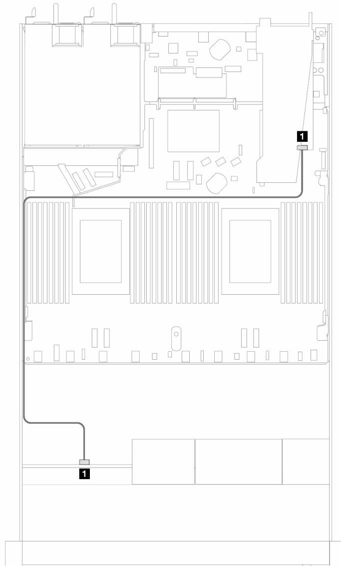
Рис. 429. Прокладка кабелей для 4 передних отсеков для 2,5-дюймовых дисков SAS/SATA с адаптером RAID 8i SFF (Gen 3/4)
