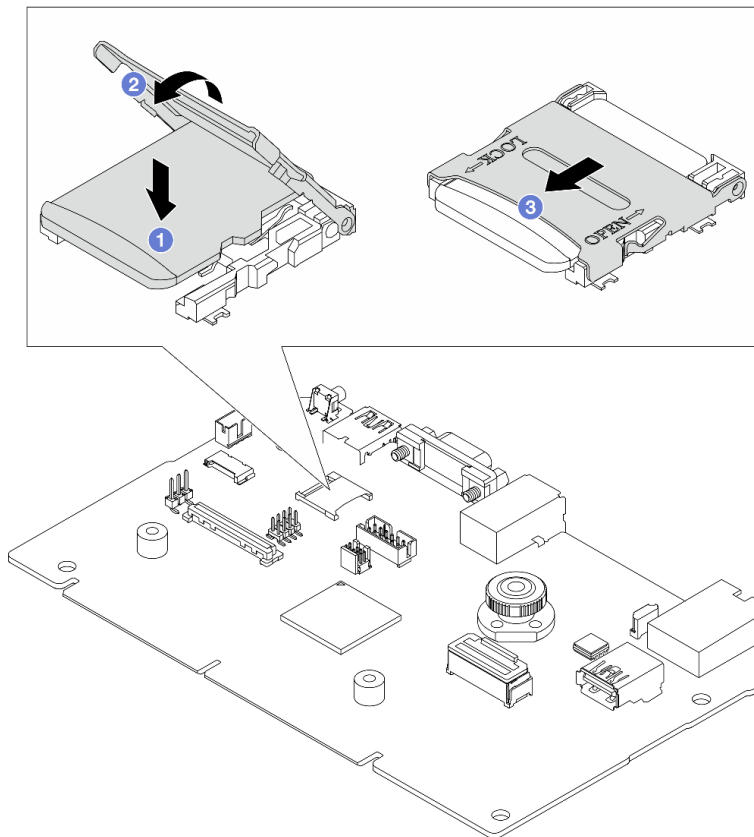
Рис. 177. Установка карты MicroSD
