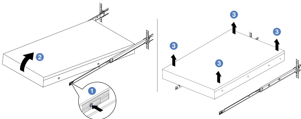
Рис. 25. Снятие сервера со стойки
