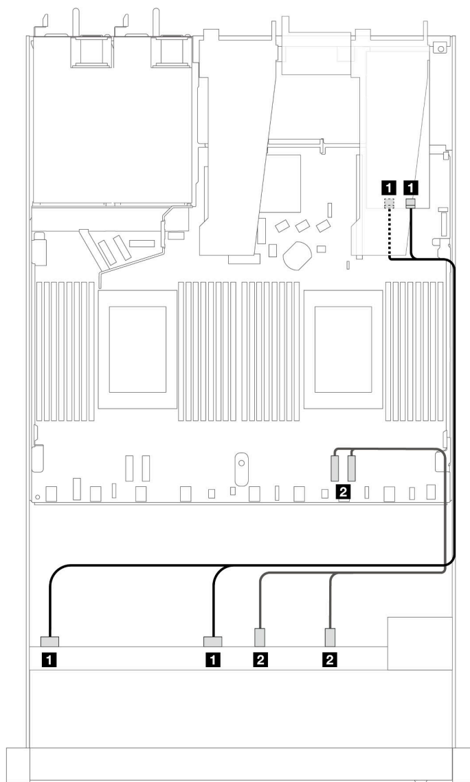
Рис. 407. Прокладка кабелей для 6 дисков SAS/SATA, 2 дисков AnyBay и 2 передних отсеков для дисков NVMe с адаптером RAID 8i или 16i SFF (Gen 3)
