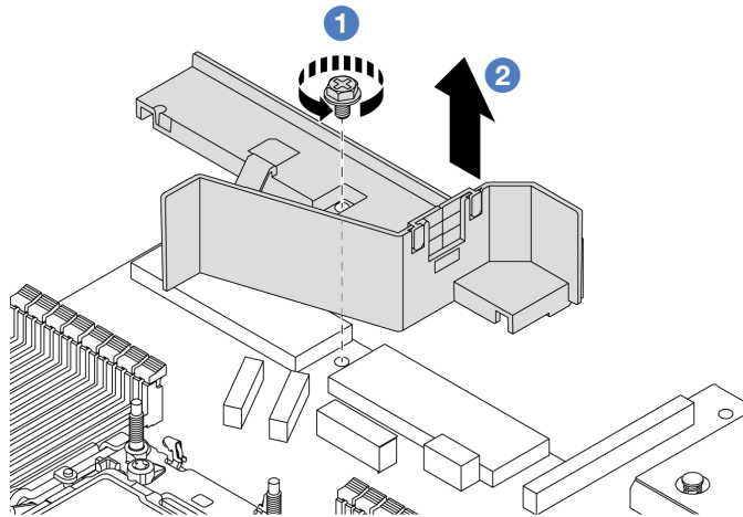
Рис. 196. Снятие дефлектора блока питания
