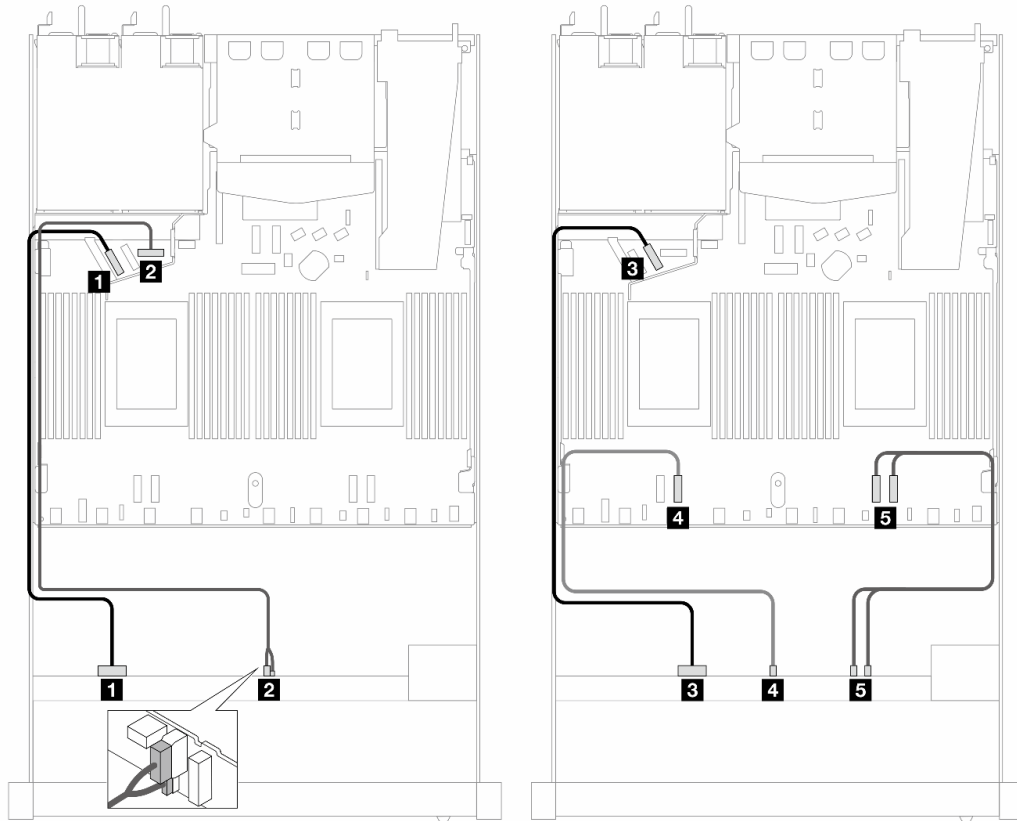
Рис. 370. Прокладка кабелей для встроенной конфигурации с 10 дисками NVMe для жидкостного охлаждения (объединительная панель Gen 5)
