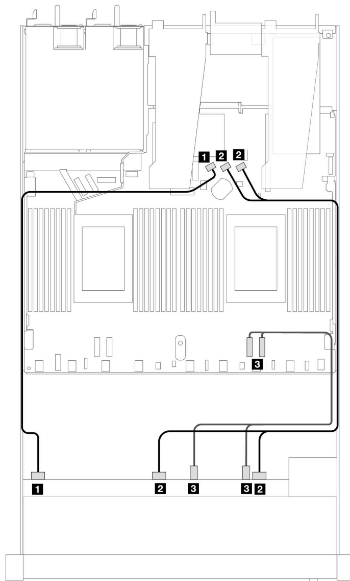
Рис. 399. Прокладка кабелей для встроенной конфигурации с шестью передними дисками SAS/SATA и четырьмя отсеками для передних дисков AduBay
