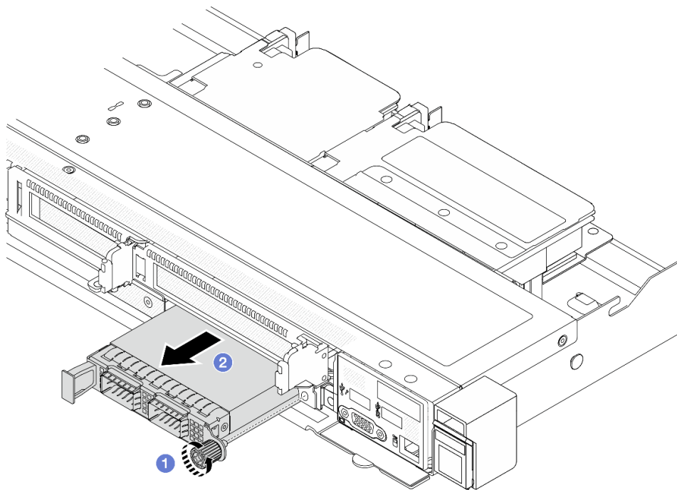
Рис. 68. Снятие переднего модуля ОСР
