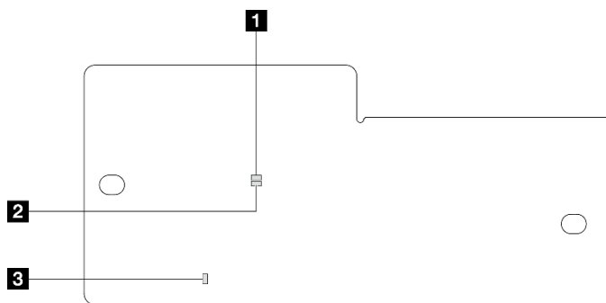
Рис. 504. Светодиодные индикаторы на компоненте «Модуль безопасности микропрограммы и RoT»
