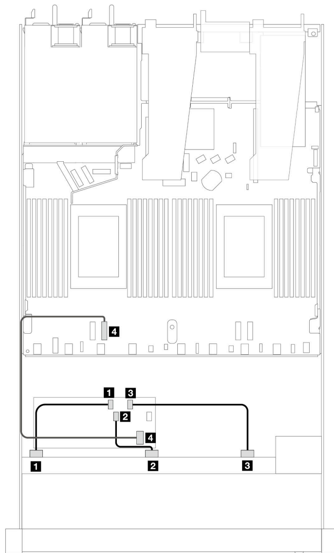
Рис. 470. Прокладка кабелей для 10 передних отсеков для дисков SAS/SATA с адаптером RAID 16i CFF (Gen 3 или Gen 4)
