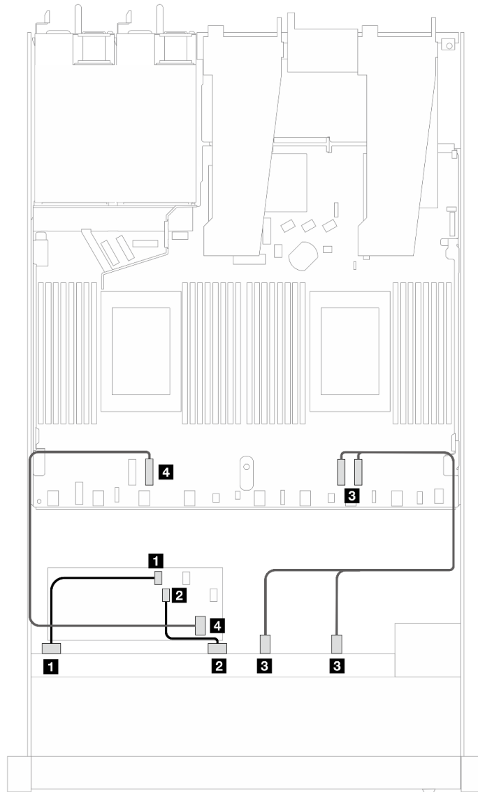
Рис. 459. Прокладка кабелей для шести передних дисков SAS/SATA и четырех отсеков для передних дисков AnyBay с адаптером RAID 16i CFF (Gen 3 или Gen 4)
