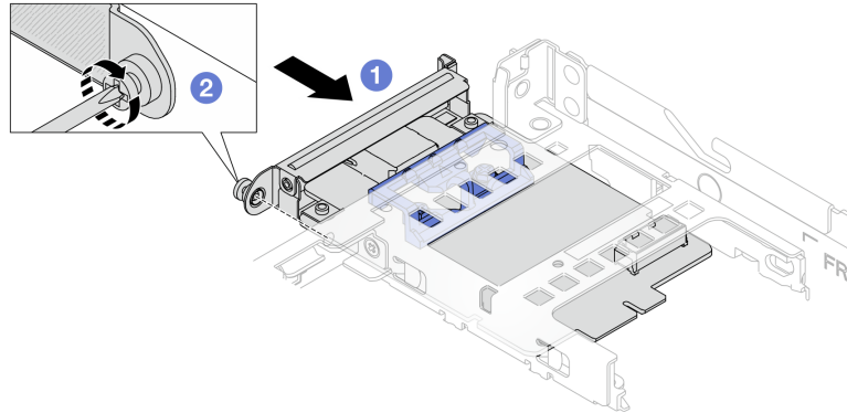
Рис. 126. Установка адаптера NIC для управления
