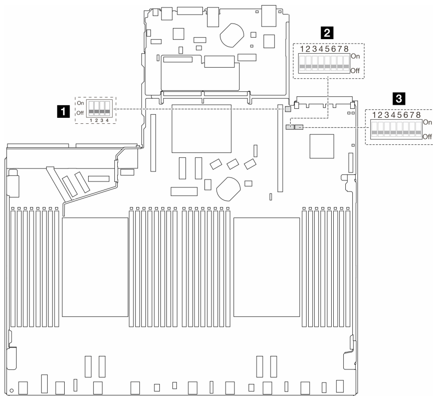
Рис. 16. Переключатели блока материнской платы
