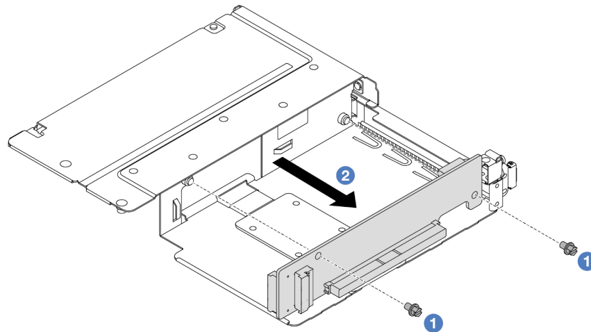
Рис. 63. Снятие платы-адаптера Riser с отсека максимальной высоты
