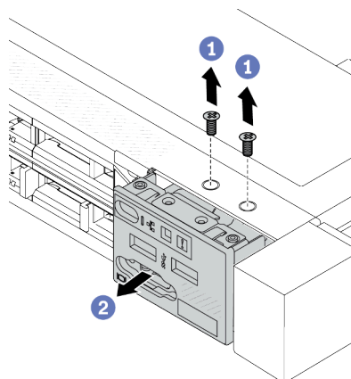
Рис. 74. Снятие переднего модуля ввода-вывода с 2,5-дюймовой рамы
