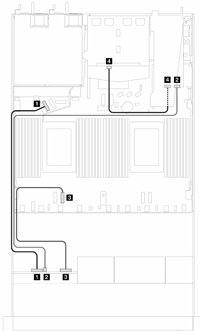
Рис. 439. Прокладка кабелей для 4 передних отсеков для 2,5-дюймовых дисков AnyBay с адаптером RAID 8i SFF (Gen 3) и 2 задних 2,5-дюймовых дисков SAS/SATA
