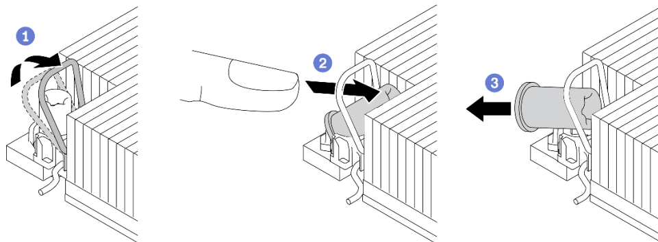
Рис. 91. Снятие гайки Torx T30 с радиатора
