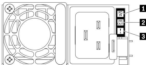
Рис. 507. Светодиодные индикаторы на модуле блока питания
