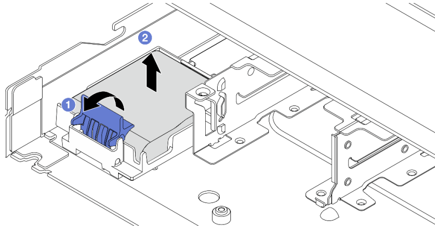
Рис. 214. Снятие модуля питания флэш-памяти RAID с рамы
