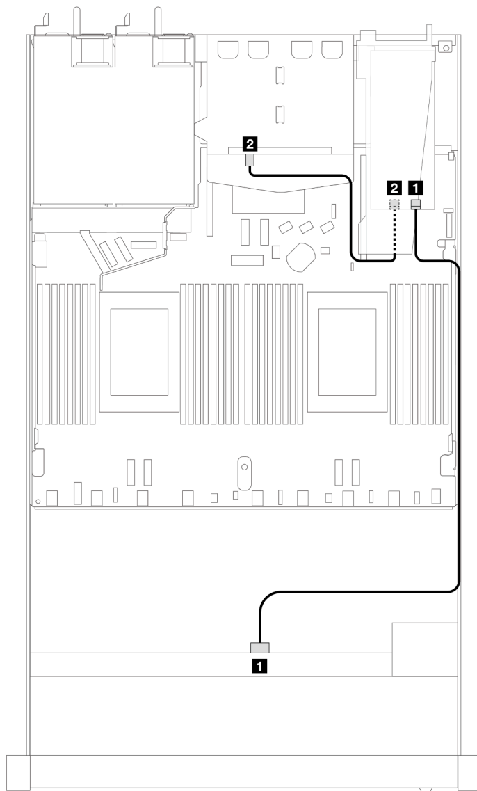
Рис. 380. Прокладка кабелей для конфигурации с четырьмя передними отсеками для 3,5-дюймовых дисков SAS/SATA, адаптером RAID 8i SFF (Gen 3) и двумя задними 2,5-дюймовыми дисками SAS/SATA
