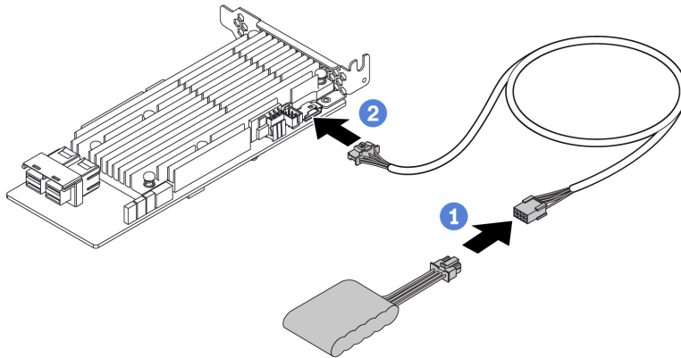
Рис. 213. Прокладка кабеля питания модуля питания флэш-памяти
