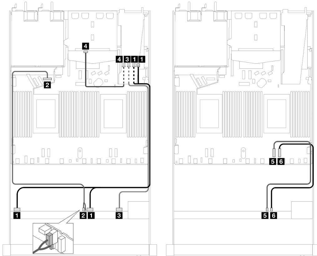
Рис. 482. Прокладка кабелей для шести передних дисков SAS/SATA, четырех отсеков для передних дисков AnyBay и адаптера RAID 16i SFF (Gen 3) при двух установленных задних дисках SAS/SATA
