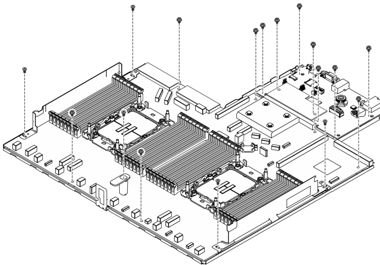
Рис. 512. Разборка блока материнской платы
