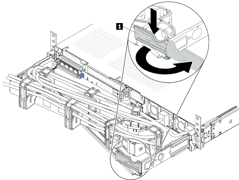
Рис. 103. Регулировка CMA
