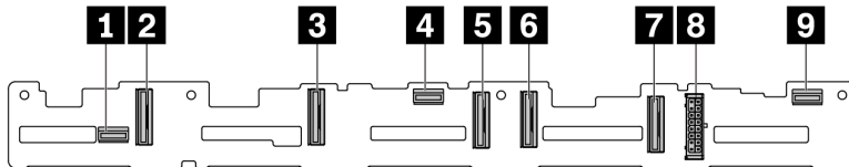
Рис. 303. Объединительная панель с 6 отсеками для дисков SAS/SATA и 4 отсеками для дисков AnyBay
