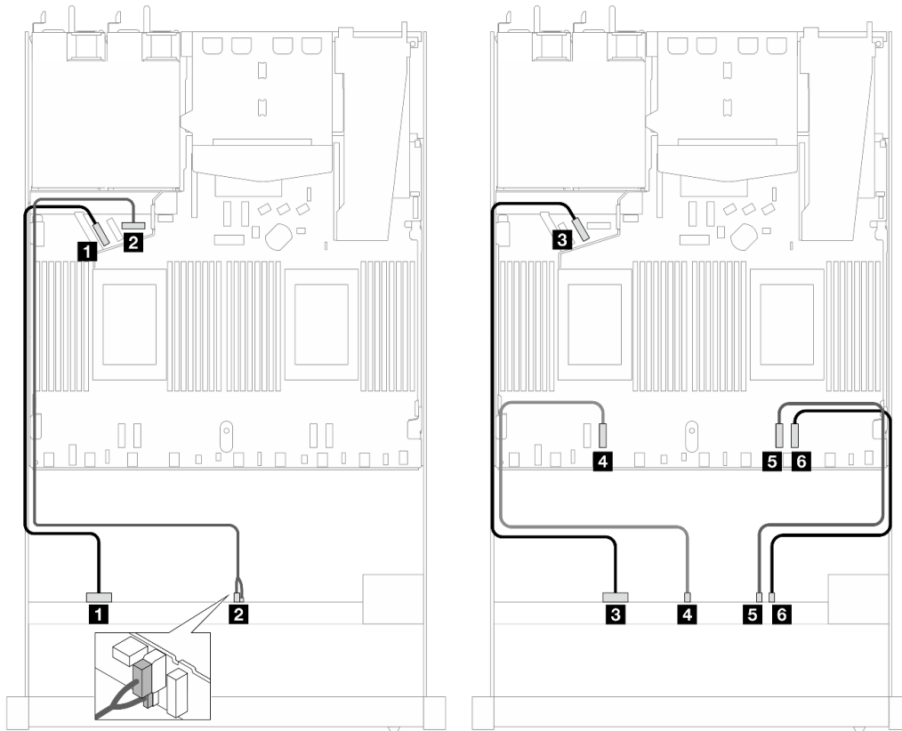
Рис. 492. Прокладка кабелей для встроенной конфигурации с 10 передними 2,5-дюймовыми дисками NVMe
