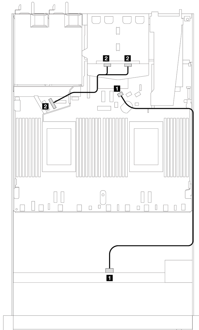
Рис. 416. Прокладка кабелей для встроенной конфигурации с четырьмя передними 3,5-дюймовыми дисками SAS/SATA и двумя задними 2,5-дюймовыми дисками NVMe
