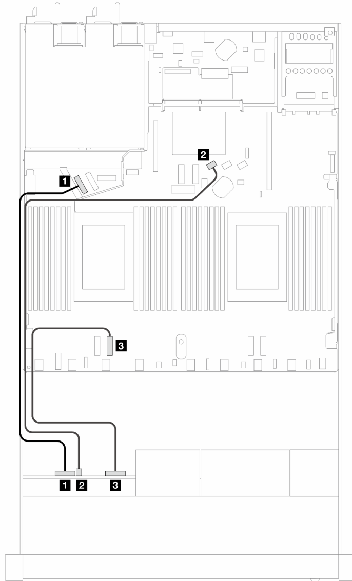
Рис. 436. Прокладка кабелей для встроенной конфигурации с 4 передними 2,5-дюймовыми дисками AduBay
