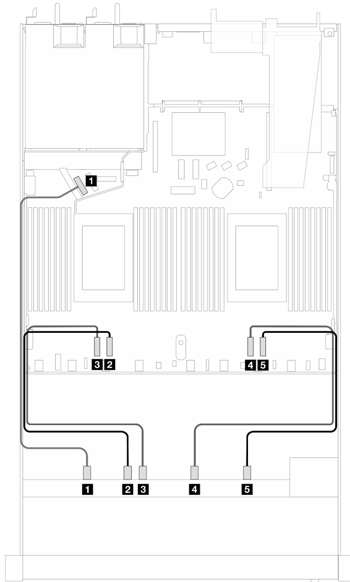
Рис. 369. Прокладка кабелей для встроенной конфигурации с 10 дисками NVMe для жидкостного охлаждения (объединительная панель Gen 4)
