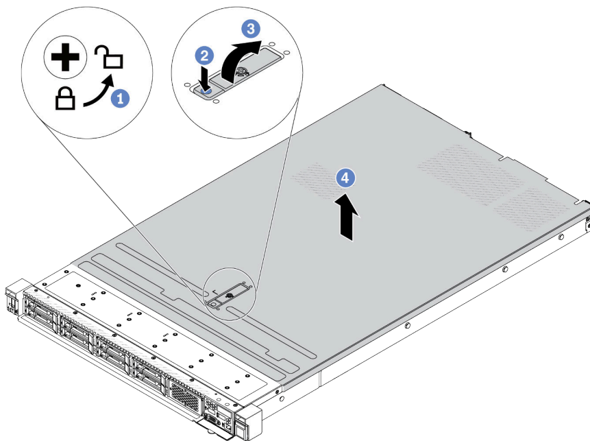
Рис. 299. Снятие верхнего кожуха
