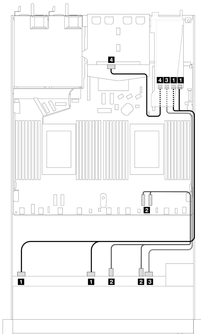
Рис. 404. Прокладка кабелей для шести передних дисков SAS/SATA, четырех отсеков для передних дисков AnyBay и адаптера RAID 16i SFF (Gen 3) с двумя установленными задними 2,5-дюймовыми дисками SAS/SATA
