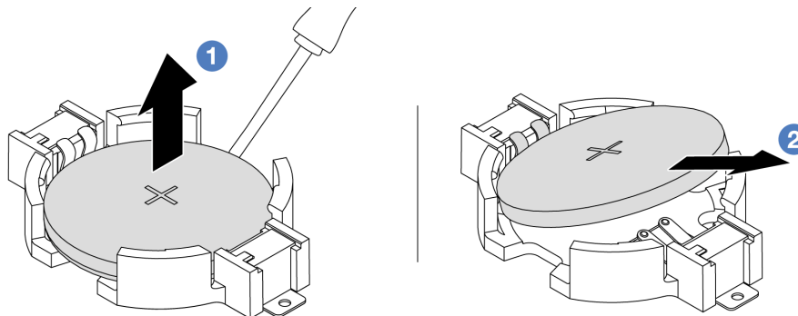
Рис. 48. Извлечение батарейки CMOS
