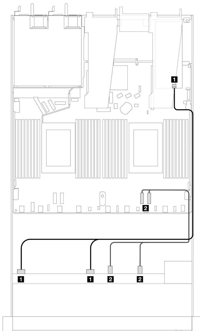
Рис. 462. Прокладка кабелей для 6 дисков SAS/SATA, 2 дисков ApyBay и 2 передних отсеков для дисков NVMe с адаптером RAID 8i или 16i SFF (Gen 4)
