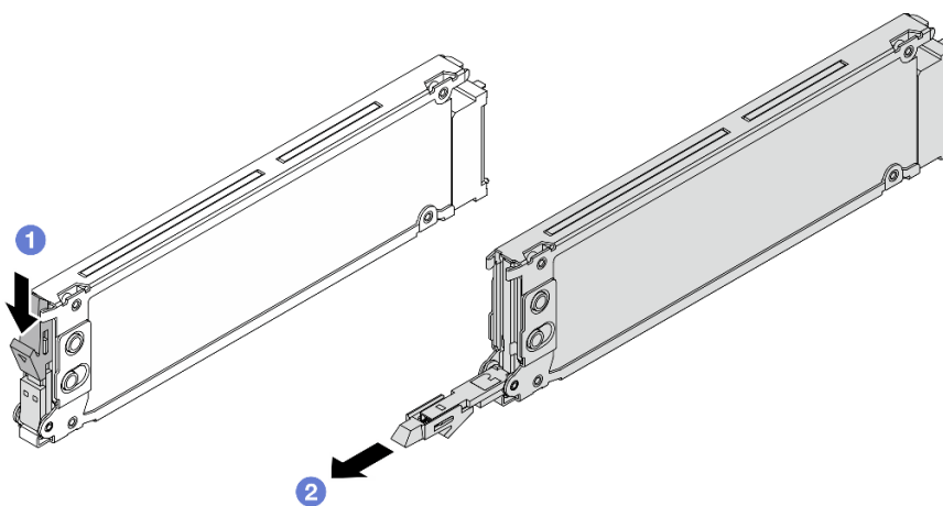
Рис. 98. Снятие диска EDSFF
