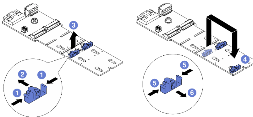
Рис. 183. Регулировка фиксатора M.2
