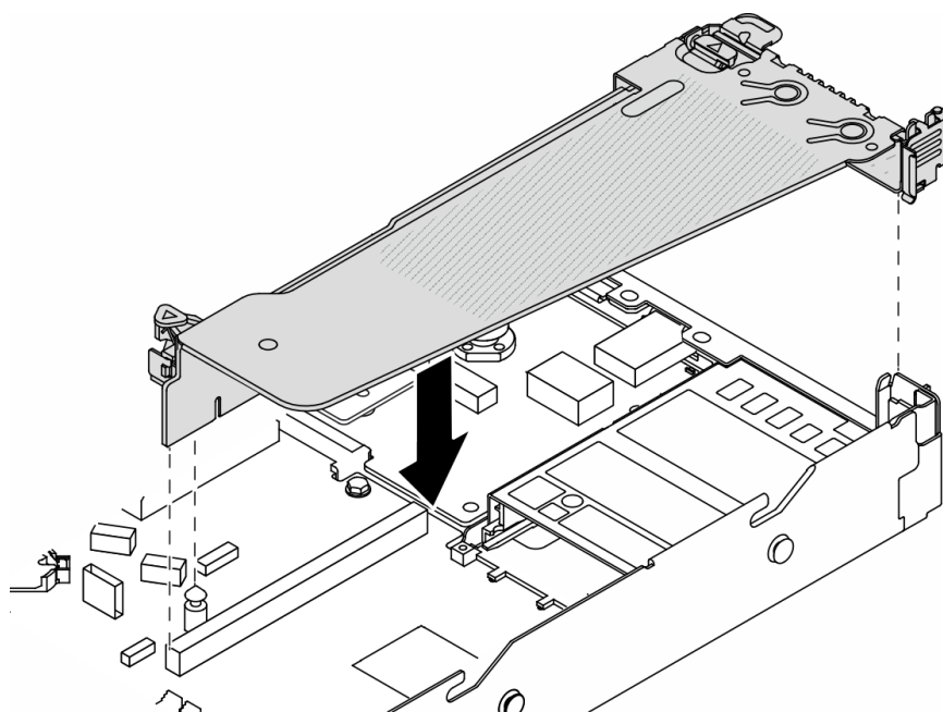
Рис. 286. Установка блока платы-адаптера Riser
