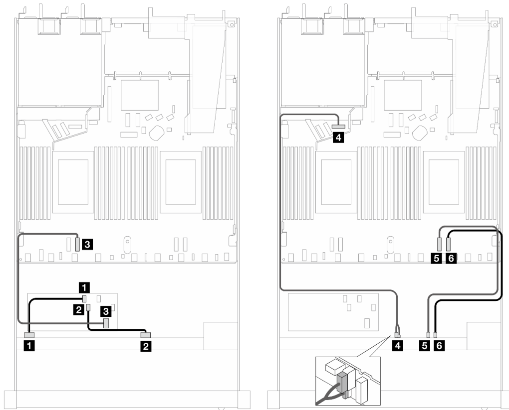
Рис. 488. Прокладка кабелей для шести дисков SAS/SATA, двух дисков AnyBay и двух передних отсеков для дисков NVMe с адаптером HBA/RAID 16i CFF (Gen 3 или Gen 4)
