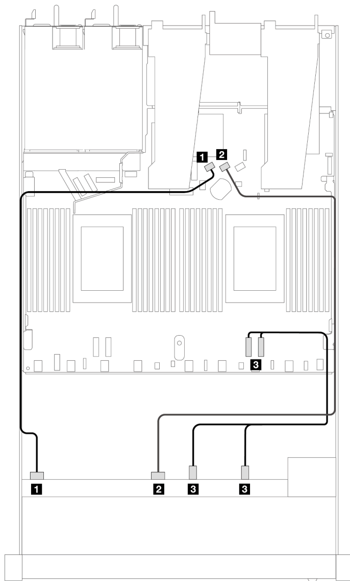
Рис. 461. Прокладка кабелей для встроенной конфигурации с шестью дисками SAS/SATA, двумя отсеками для передних дисков APU Bay и двумя отсеками для передних дисков NVMe
