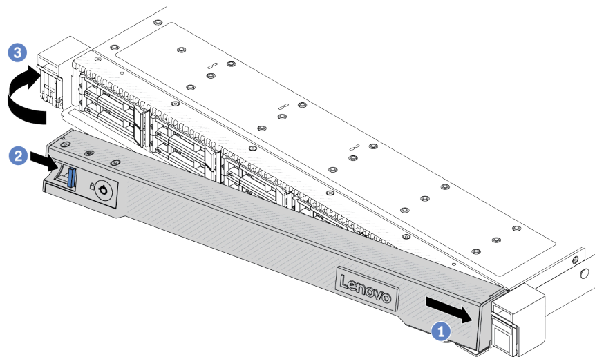
Рис. 279. Установка защитной панели
