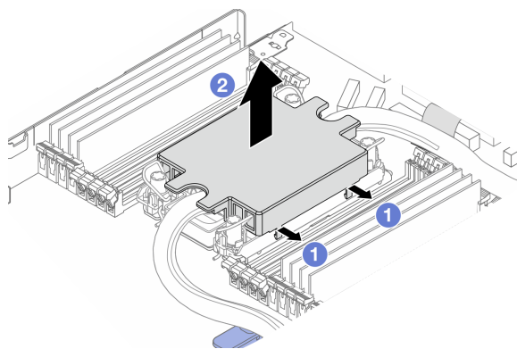
Рис. 511. Снятие кожуха платы охлаждения
