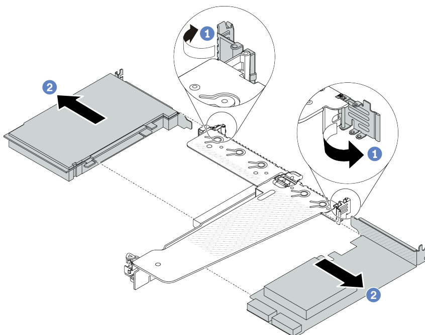
Рис. 194. Снятие адаптера PCIe с блока платы-адаптера Riser LP-FH
