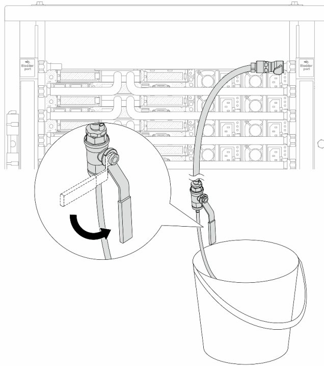
Рис. 153. Открытие клапана отводной трубки на стороне возврата
