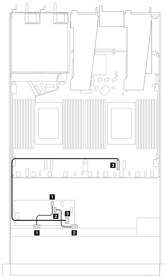
Рис. 394. Прокладка кабелей для 8 передних отсеков для 2,5-дюймовых дисков SAS/SATA и адаптера RAID 8i или 16i CFF (Gen 3)
