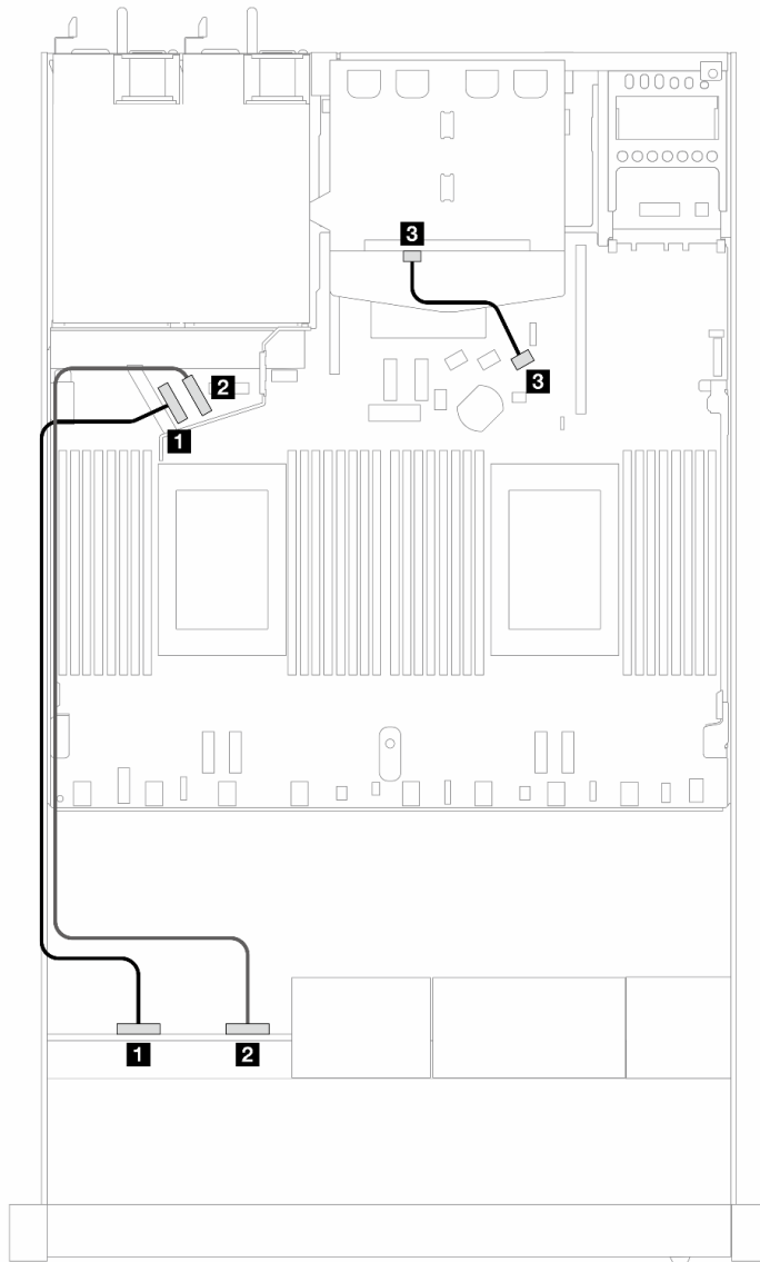
Рис. 435. Прокладка кабелей для встроенной конфигурации с 4 передними 2,5-дюймовыми дисками NVMe и 2 задними 2,5-дюймовыми дисками SAS/SATA
