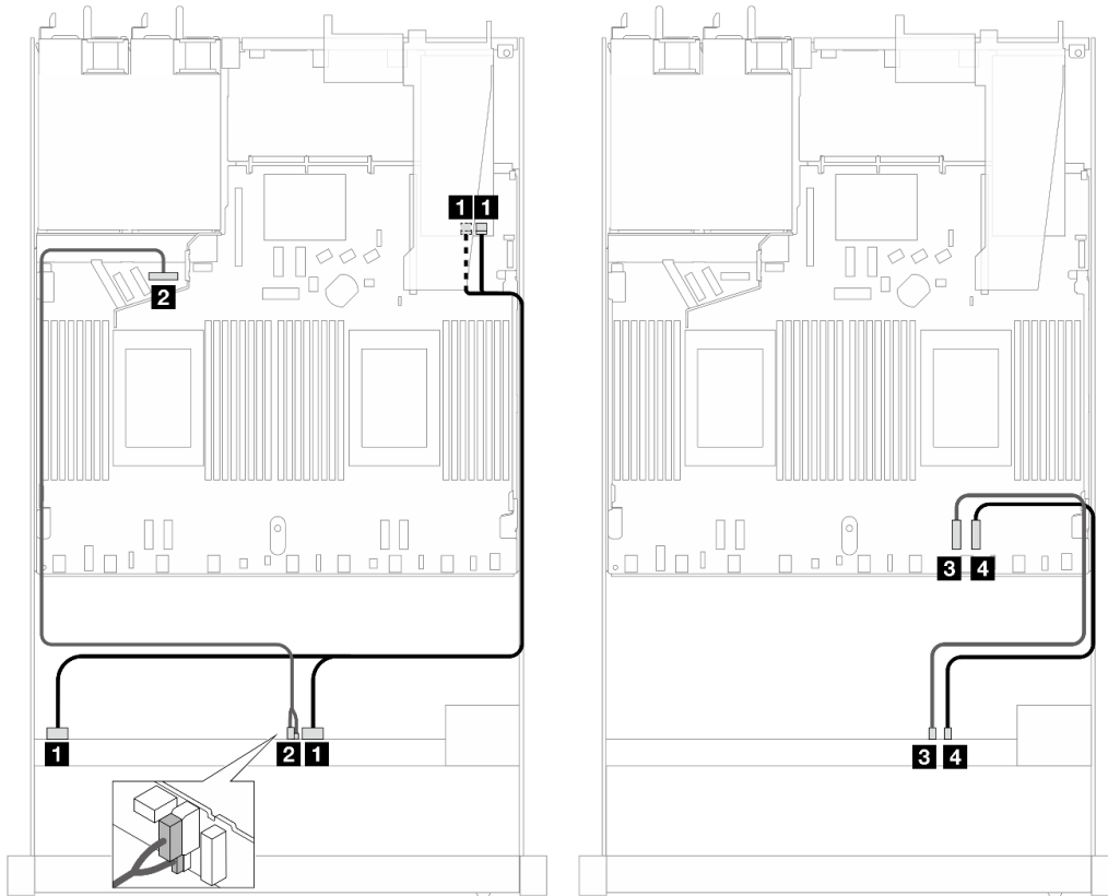
Рис. 487. Прокладка кабелей для шести дисков SAS/SATA, двух дисков AnyBay и двух передних отсеков для дисков NVMe с адаптером RAID 16i SFF (Gen 3)
