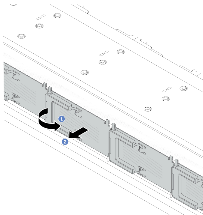
Рис. 97. Снятие кожуха отсека для дисков EDSFF
