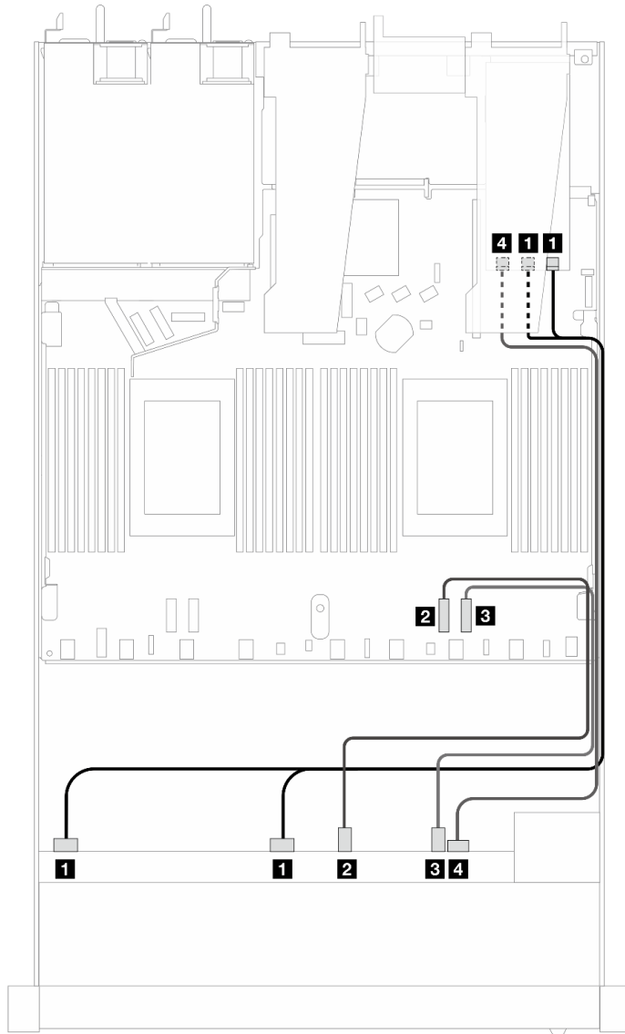
Рис. 357. Прокладка кабелей для шести передних дисков SAS/SATA и четырех отсеков для передних дисков AnyBay с адаптером RAID 8i или 16i SFF (Gen 3)
