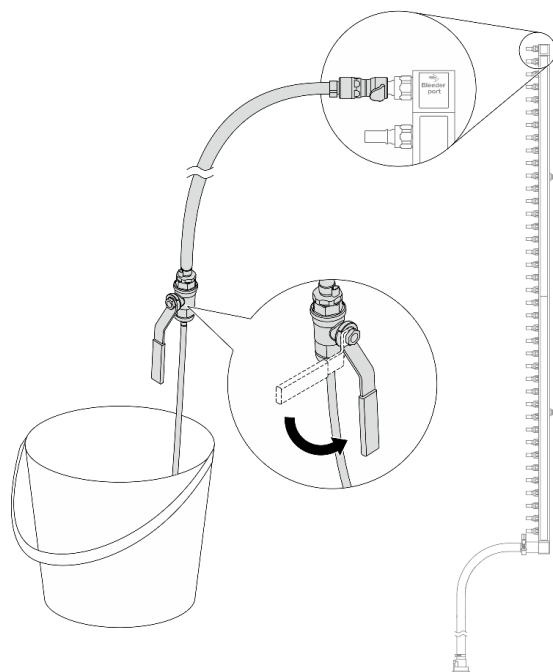
Рис. 161. Открытие клапана отводной трубки
