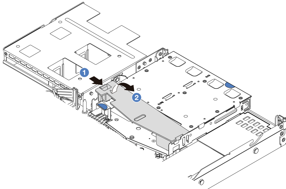
Рис. 39. Снятие дефлектора
