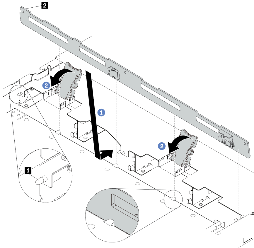
Рис. 36. Установка объединительной панели для четырех 3,5-дюймовых оперативно заменяемых дисков
