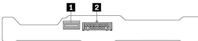
Рис. 314. Задняя объединительная панель с 2 отсеками для 2,5-дюймовых дисков NVMe
