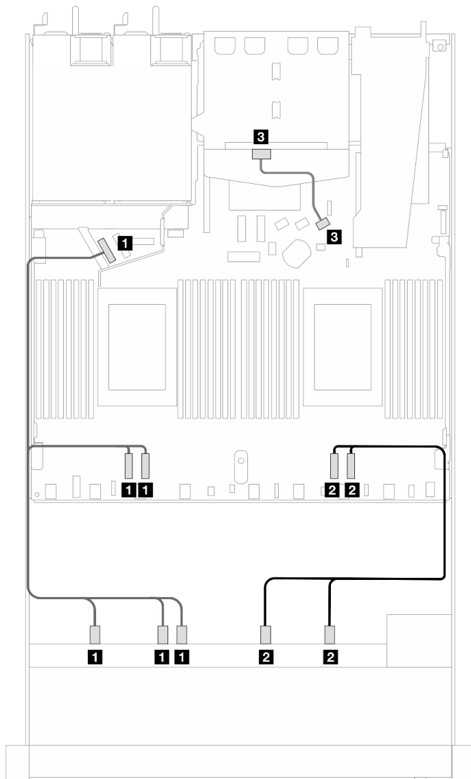
Рис. 477. Прокладка кабелей для встроенной конфигурации с 10 передними 2,5-дюймовыми дисками NVMe и двумя установленными задними 2,5-дюймовыми дисками SAS/SATA
