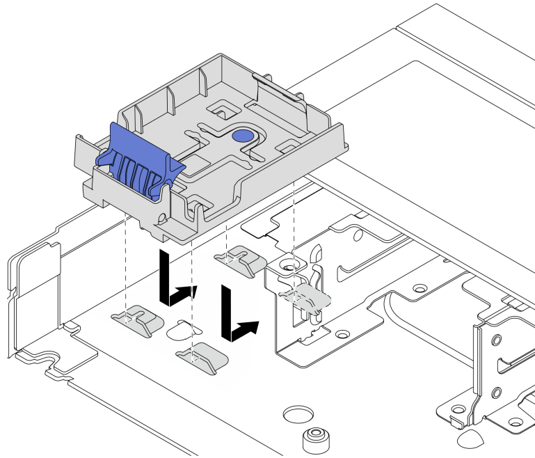
Рис. 217. Установка держателя модуля питания флэш-памяти RAID
