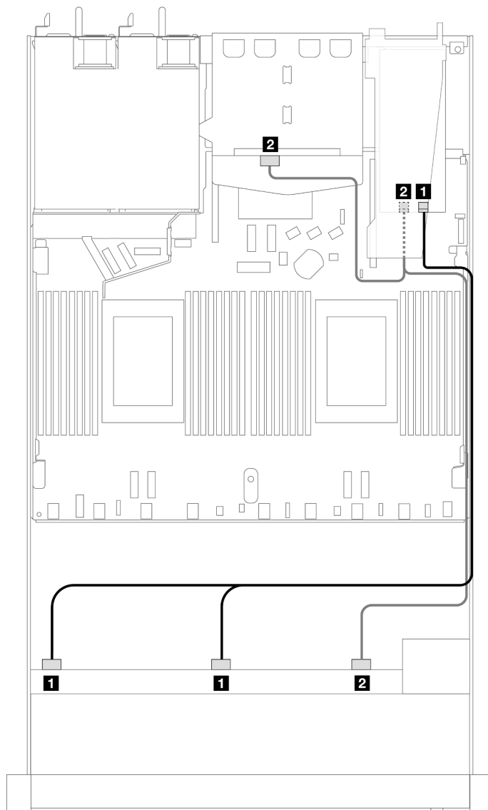
Рис. 410. Прокладка кабелей для 10 передних отсеков для дисков SAS/SATA и адаптера RAID 16i SFF (Gen 4) с двумя установленными задними 2,5-дюймовыми дисками SAS/SATA
