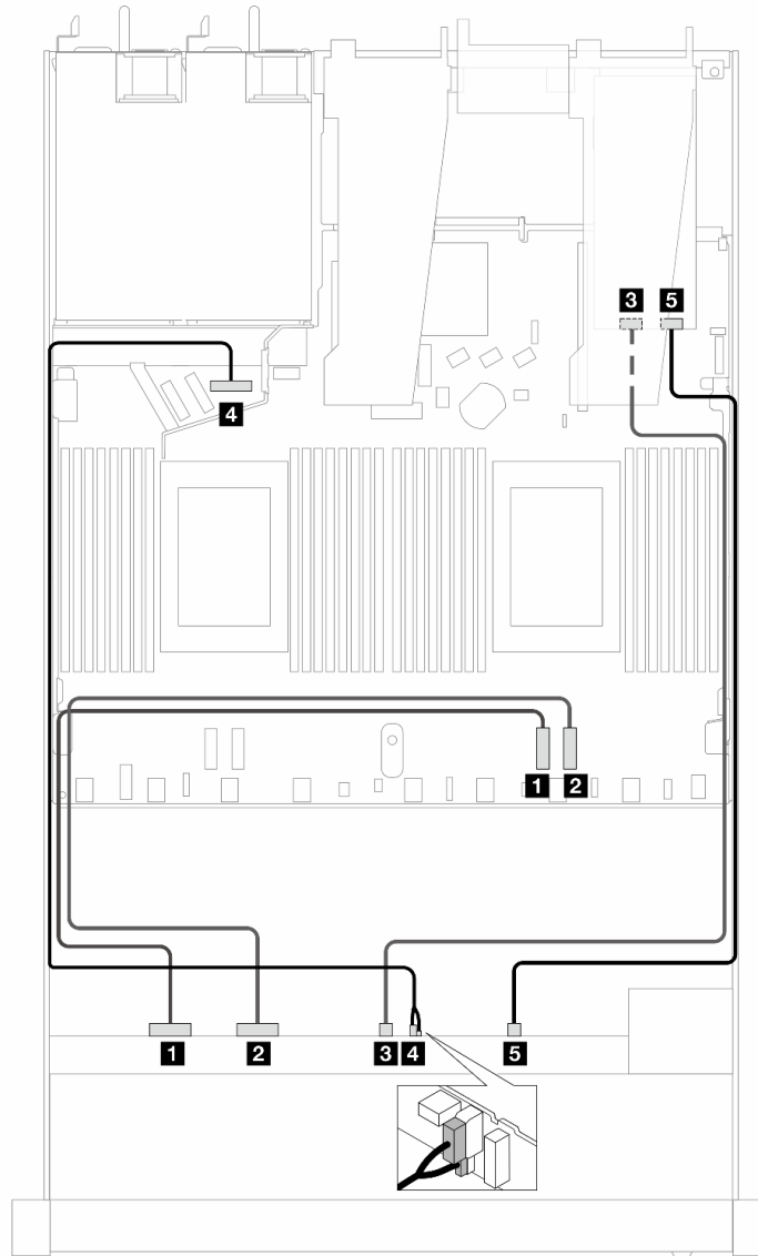
Рис. 364. Прокладка кабелей восьми передних дисков U.2 для подключения к встроенным разъемам и адаптеру ретаймера SFF Gen 5
