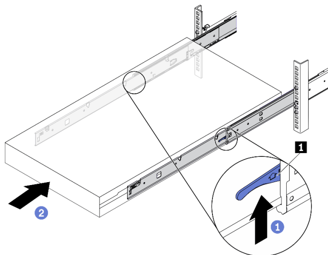
Рис. 28. Установка сервера в стойку
