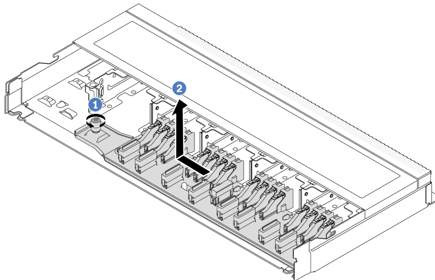
Рис. 37. Снятие объединительной панели с 16 отсеками для дисков EDSFF
