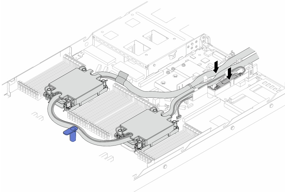
Рис. 122. Размещение шлангов и модуля
