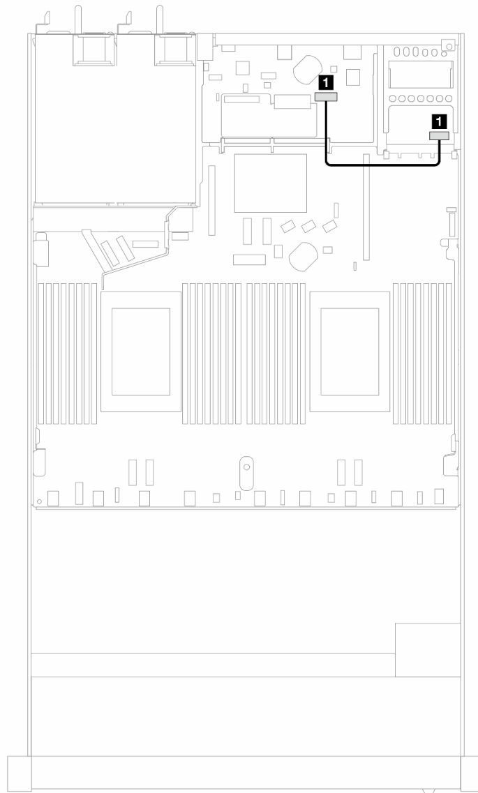
Рис. 337. Прокладка кабелей для адаптера NIC для управления
