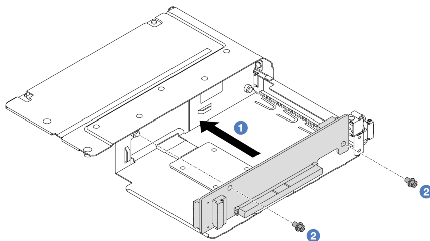
Рис. 65. Установка платы-адаптера Riser в отсек максимальной высоты
