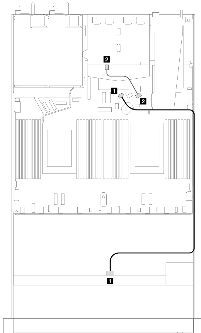
Рис. 378. Прокладка кабелей для встроенной конфигурации с четырьмя передними отсеками для 3,5-дюймовых дисков SAS/SATA и двумя задними 2,5-дюймовыми дисками SAS/SATA
