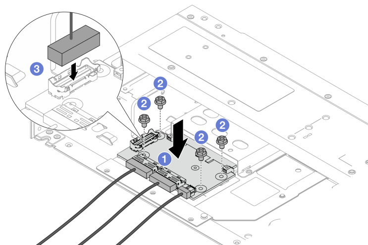
Рис. 71. Установка передней карты интерпозера OCP
