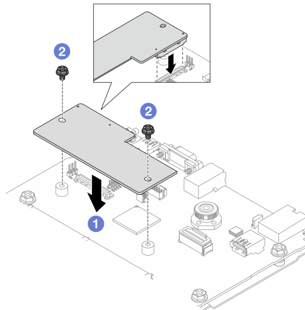
Рис. 289. Установка Модуль безопасности микропрограммы и RoT
