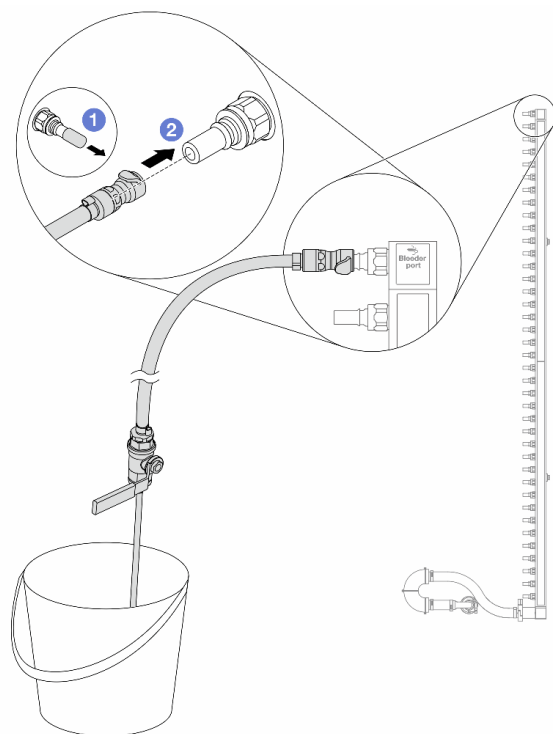
Рис. 139. Установка комплекта отводной трубки на стороне возврата
