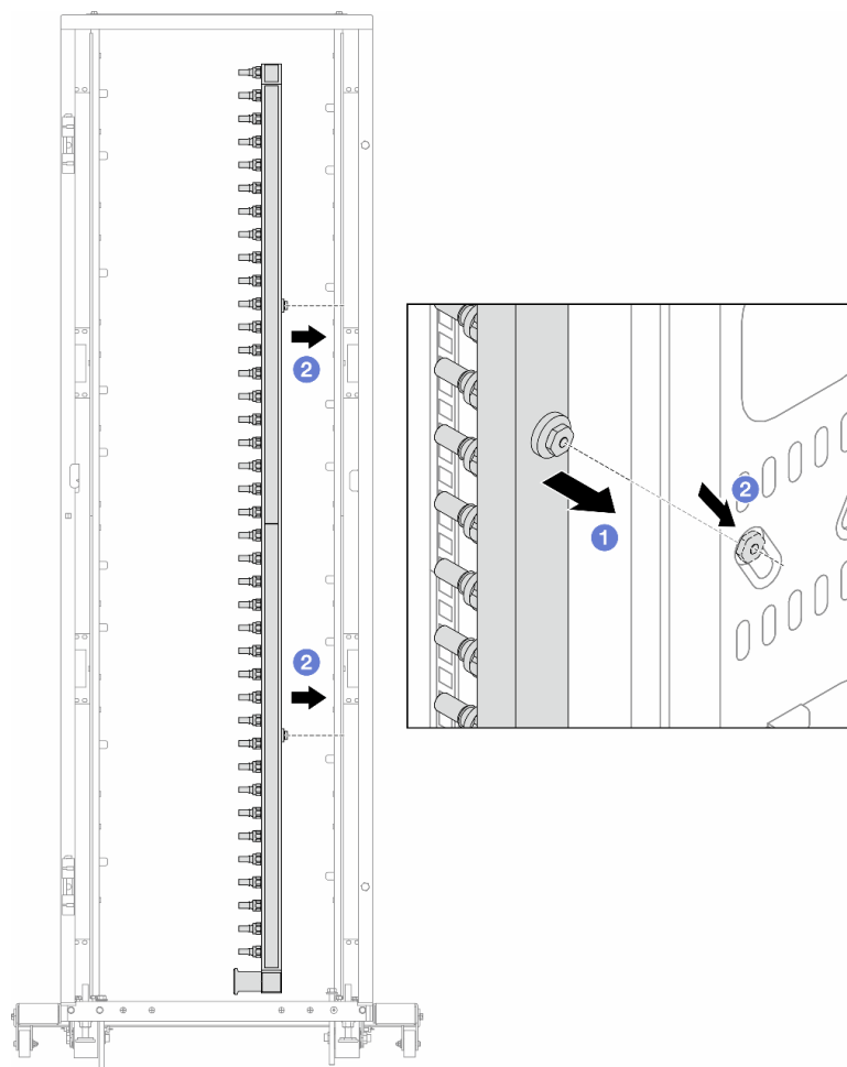
Рис. 163. Установка коллектора
