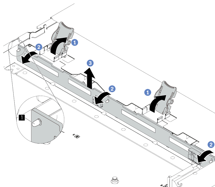
Рис. 35. Снятие объединительной панели для 3,5-дюймовых дисков
