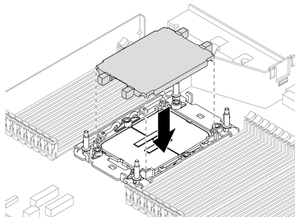
Рис. 118. Установка кожуха гнезда процессора
