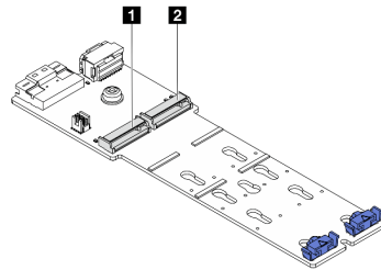
Рис. 184. Гнездо для диска M.2
