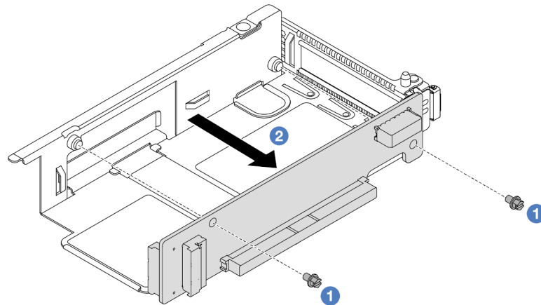
Рис. 62. Снятие платы-адаптера Riser с низкопрофильного отсека
