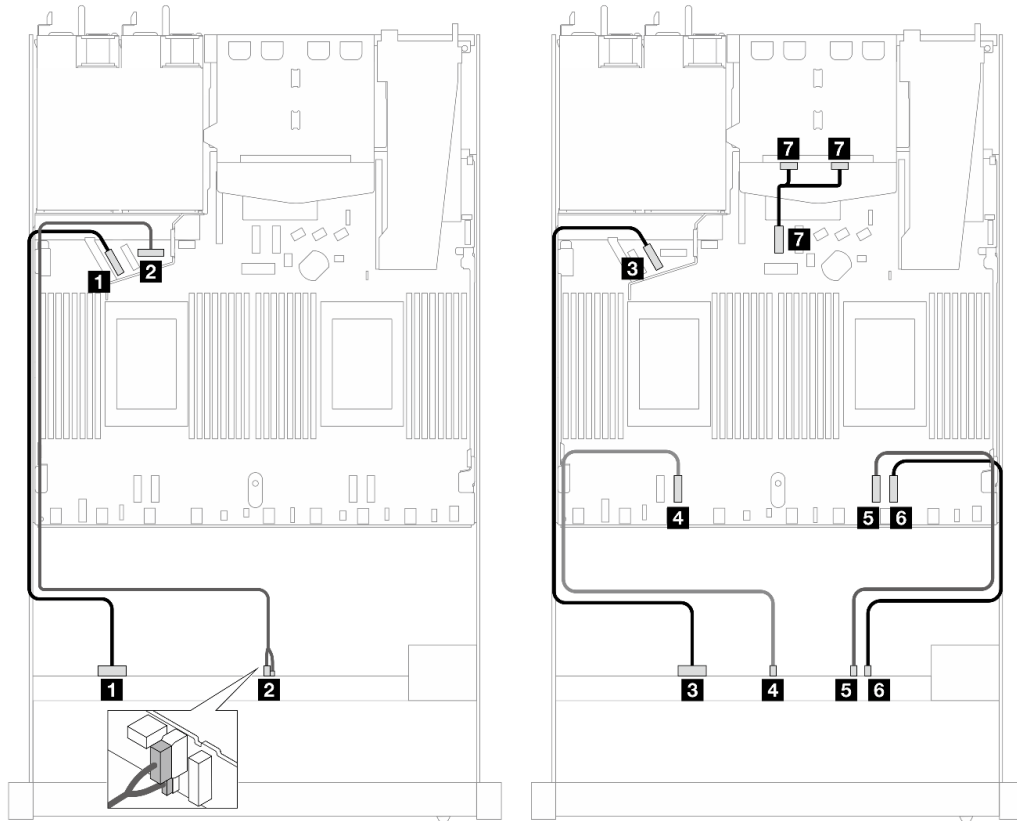
Рис. 493. Прокладка кабелей для встроенной конфигурации с 12 передними 2,5-дюймовыми дисками NVMe
