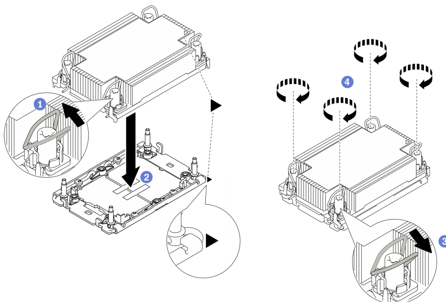
Рис. 208. Установка модуля РНМ
