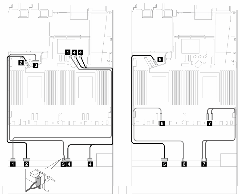
Рис. 371. Прокладка кабелей для встроенной конфигурации с 10 передними дисками AлуВау (объединительная панель Gen 5)
