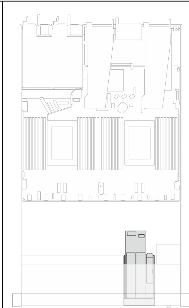
Рис. 339. Блок дисков M.2 на раме с 16 отсеками для дисков EDSFF
