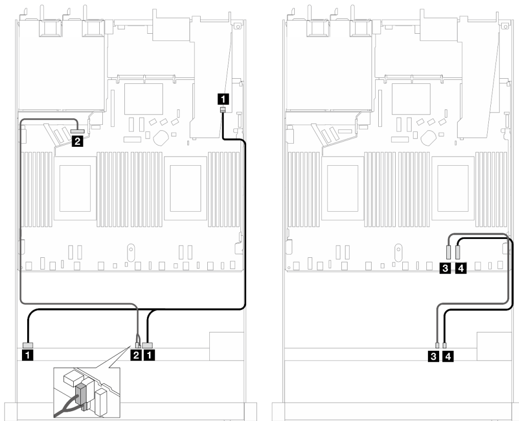
Рис. 486. Прокладка кабелей для шести дисков SAS/SATA, двух дисков AnyBay и двух передних отсеков для дисков NVMe с адаптером RAID 16i SFF (Gen 4)
