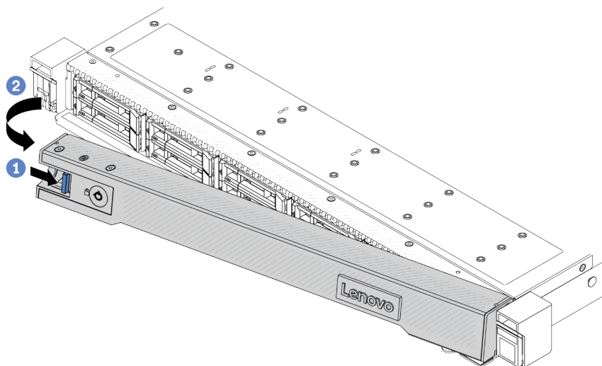
Рис. 277. Снятие защитной панели
