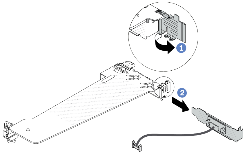
Рис. 282. Снятие скобы платы-адаптера Riser
