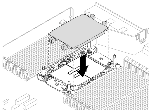
Рис. 110. Установка кожуха гнезда процессора
