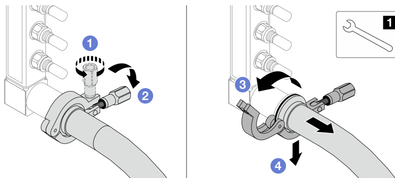
Рис. 162. Отделение коллектора от комплекта шланга
