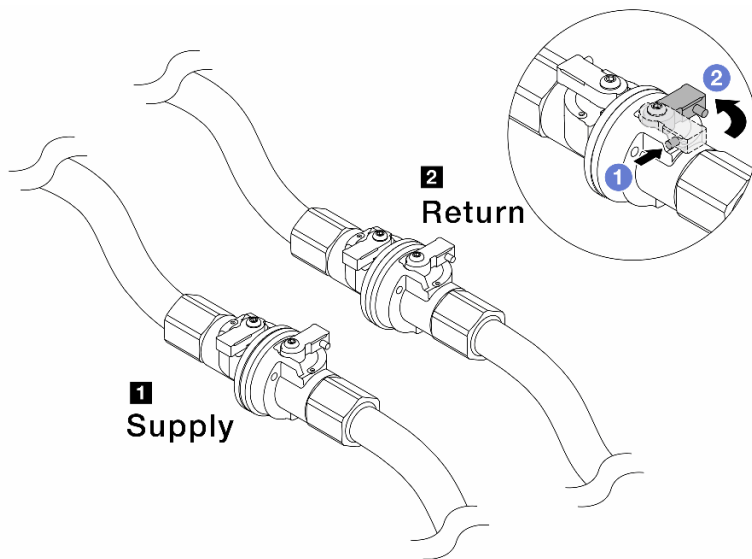
Рис. 155. Закрытие шаровых клапанов
