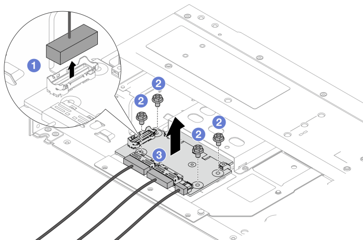
Рис. 70. Снятие передней карты интерпозера OCP
