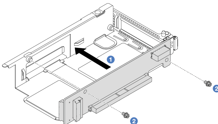
Рис. 64. Установка платы-адаптера Riser в низкопрофильный отсек
