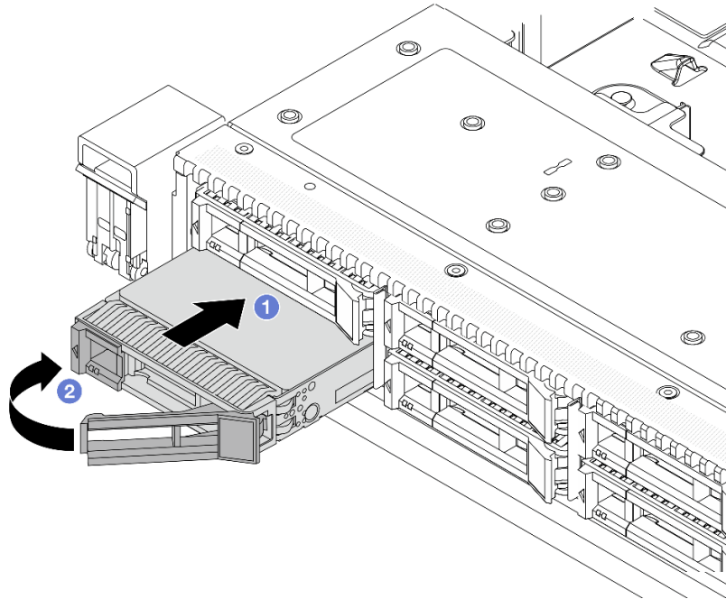
Рис. 96. Установка оперативно заменяемого диска
