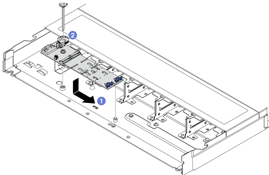
Рис. 185. Установка объединительной панели M.2
