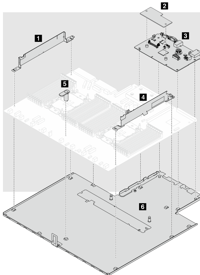
Рис. 514. Разборка блока материнской платы
