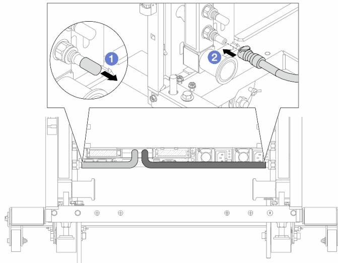
Рис. 148. Установка быстроразъемного соединителя
