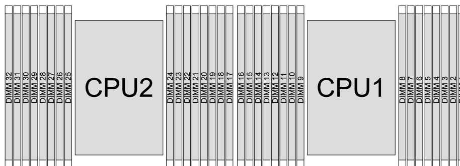
Рис. 21. Гнезда модулей памяти на процессорной плате
