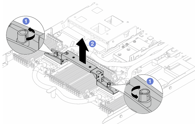
Рис. 120. Снятие ручки модуля
