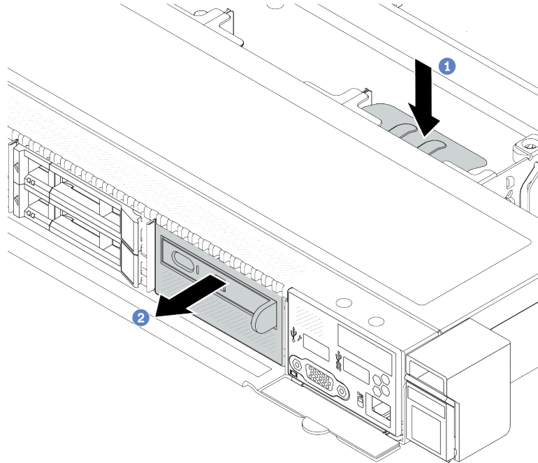
Рис. 78. Снятие блока встроенной панели диагностики
