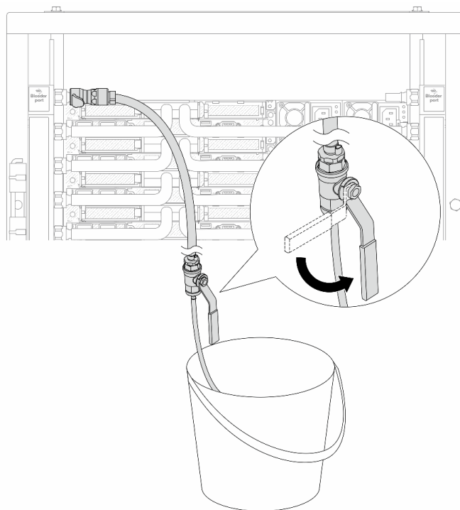
Рис. 154. Открытие клапана отводной трубки на стороне подачи
