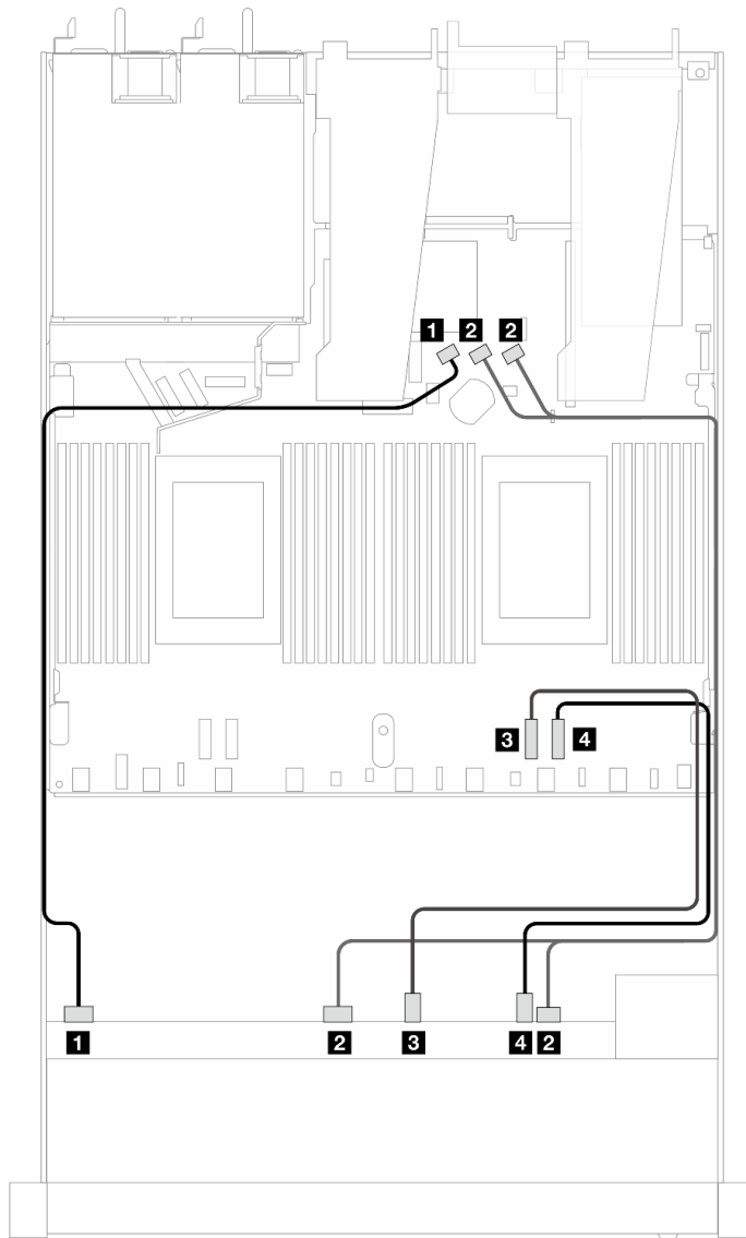
Рис. 353. Прокладка кабелей для встроенной конфигурации с шестью передними дисками SAS/SATA и четырьмя передними дисками NVMe
