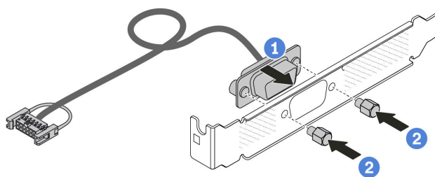
Рис. 284. Сборка модуля последовательного порта
