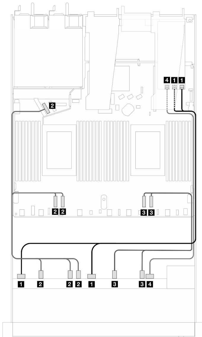
Рис. 474. Прокладка кабелей для 10 дисков AnyBay с адаптером RAID 16i SFF (Gen 3)
