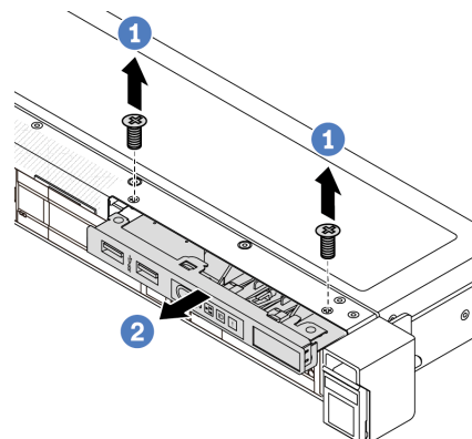
Рис. 75. Снятие переднего модуля ввода-вывода с 3,5-дюймовой рамы
