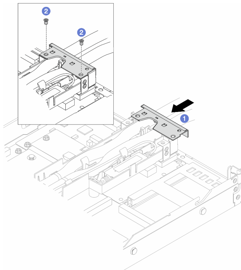
Рис. 124. Установка кожуха
