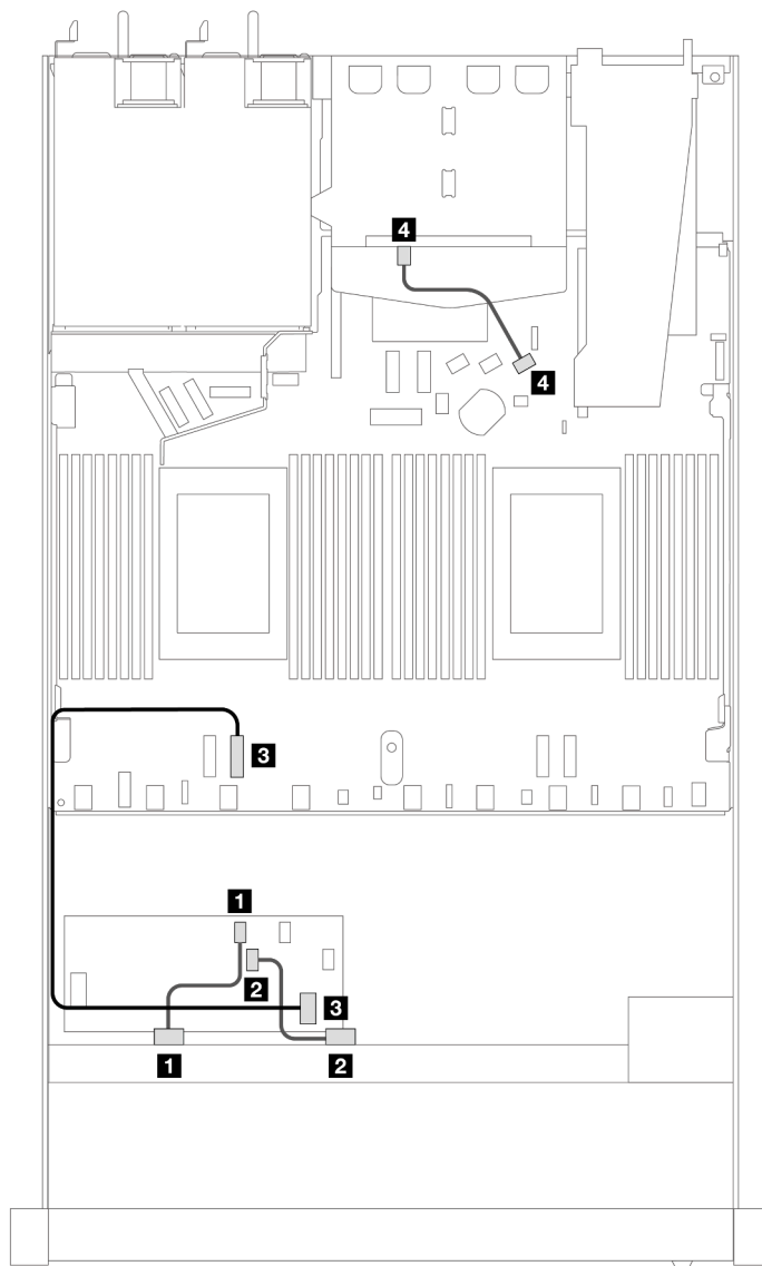
Рис. 450. Прокладка кабелей для 8 передних отсеков для 2,5-дюймовых дисков SAS/SATA, адаптера RAID 8i CFF (Gen 3) и 2 установленных 2,5-дюймовых дисков SAS/SATA
