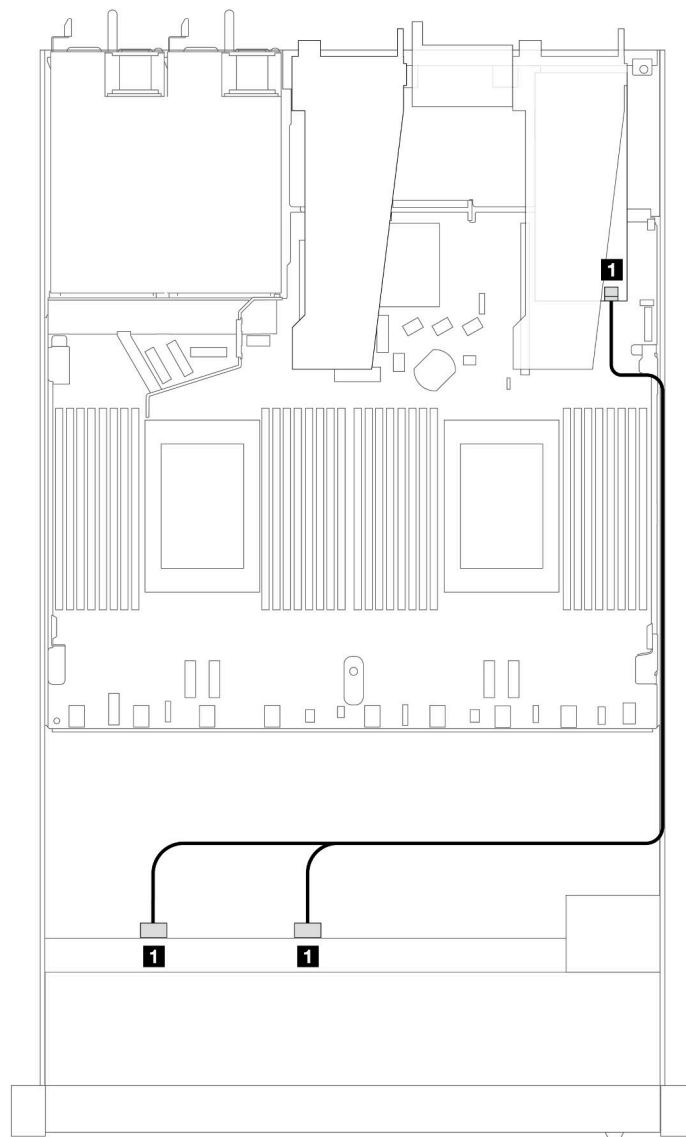
Рис. 362. Прокладка кабелей для 8 передних отсеков для 2,5-дюймовых дисков SAS/SATA и адаптера RAID 8i SFF (Gen 4)
