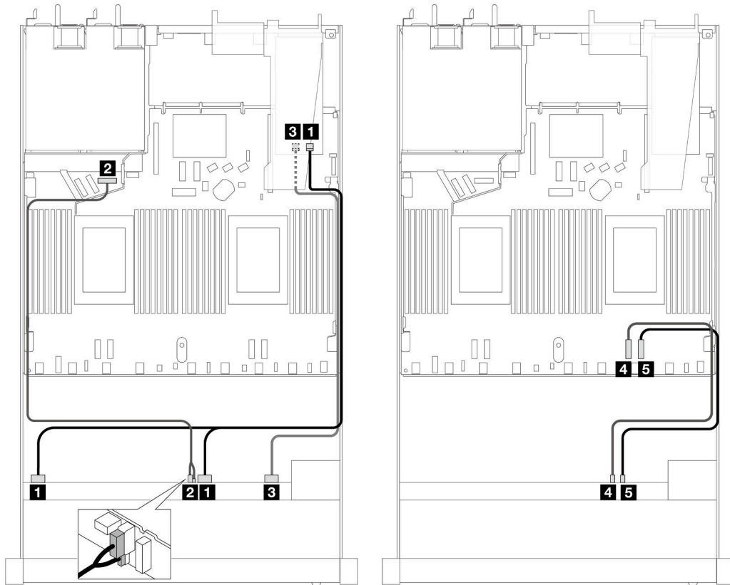
Рис. 479. Прокладка кабелей для шести передних дисков SAS/SATA и четырех отсеков для передних дисков AnyBay с адаптером RAID 16i SFF (Gen 4)
