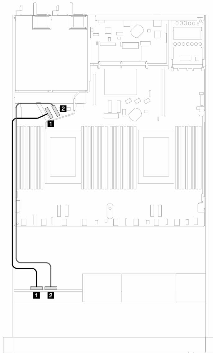
Рис. 432. Прокладка кабелей для встроенной конфигурации с 4 передними 2,5-дюймовыми дисками NVMe
