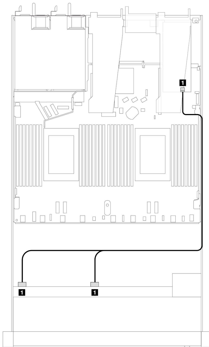
Рис. 397. Прокладка кабелей для 8 передних 2,5-дюймовых дисков U.3 с адаптером RAID 8i SFF (Gen 4)
