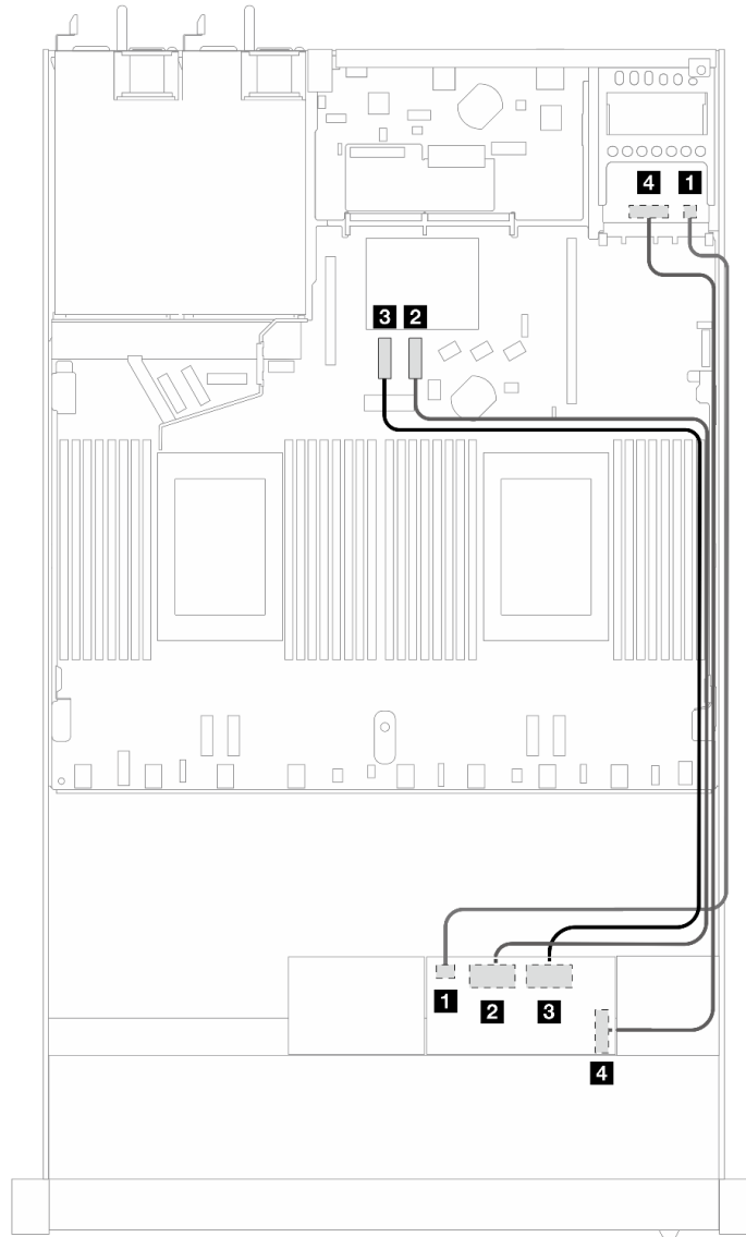
Рис. 331. Прокладка кабелей для карт интерпозера OCP
