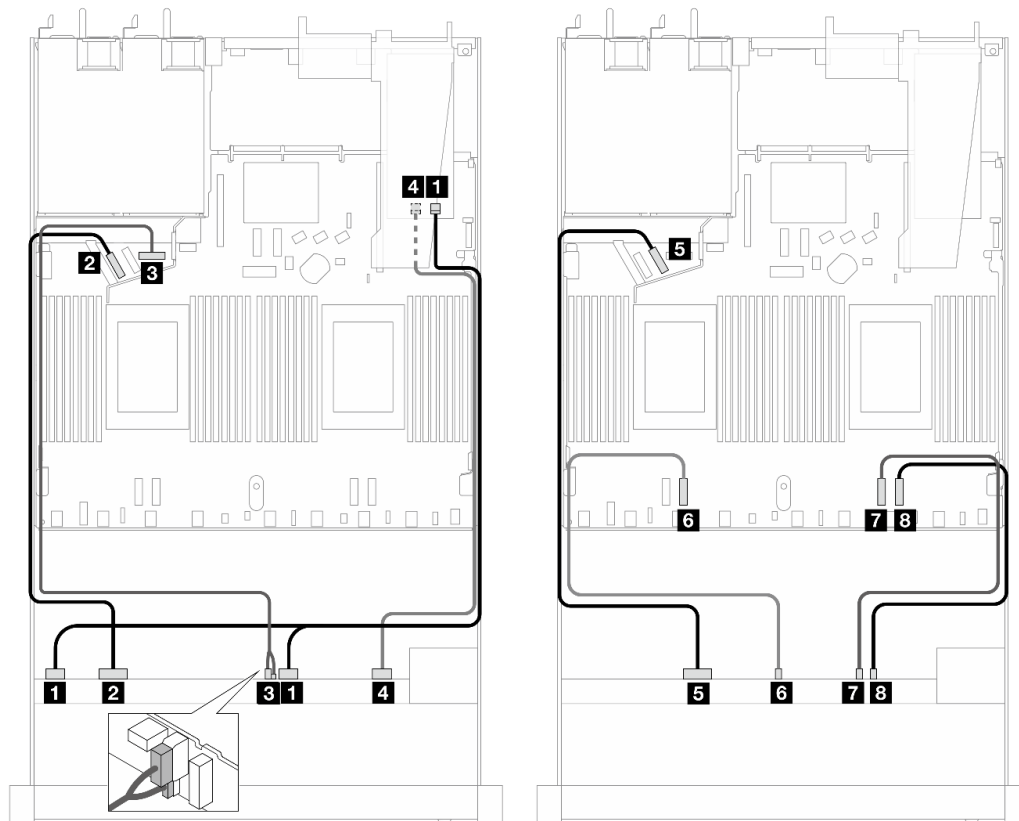
Рис. 490. Прокладка кабелей для 10 передних дисков AnyBay с адаптером RAID 16i SFF (Gen 4)
