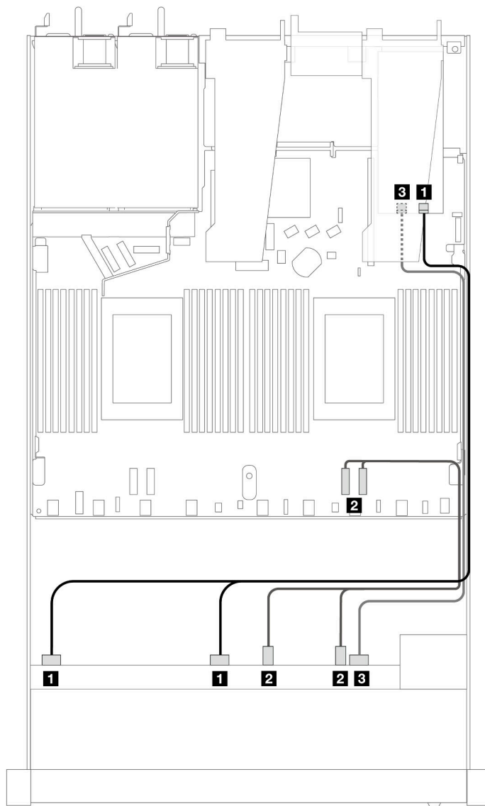
Рис. 455. Прокладка кабелей для шести передних дисков SAS/SATA и четырех отсеков для передних дисков AnyBay с адаптером RAID 16i SFF (Gen 4)
