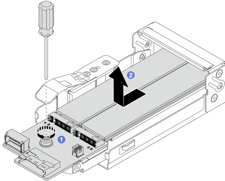
Рис. 191. Снятие объединительной панели M.2
