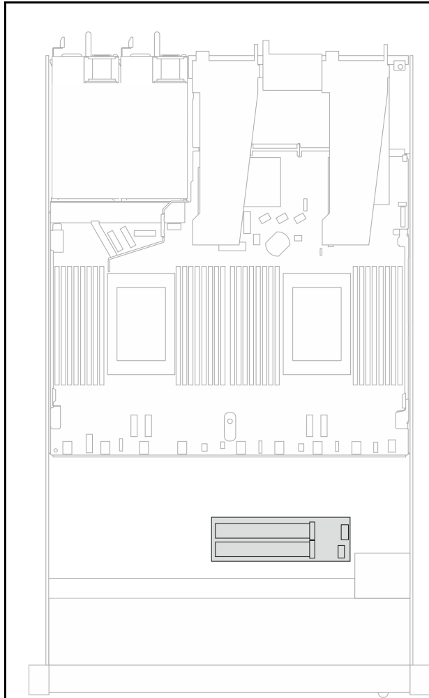
Рис. 338. Блок дисков M.2 на раме для 2,5-дюймовых и 3,5-дюймовых дисков
