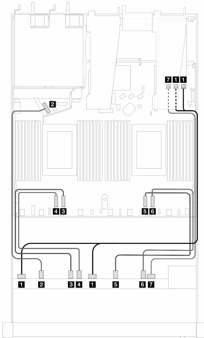
Рис. 376. Прокладка кабелей для 10 дисков AnyBay с адаптером RAID 16i SFF (Gen 3)
