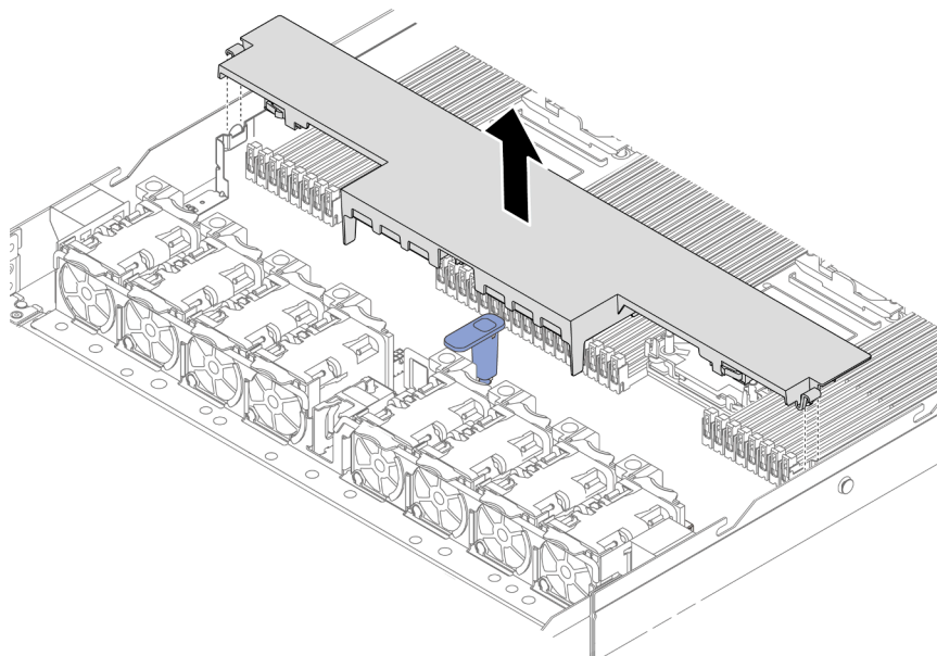
Рис. 31. Снятие дефлектора
