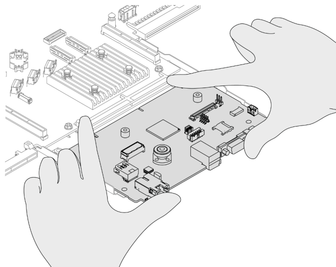
Рис. 292. Установка обеими руками
