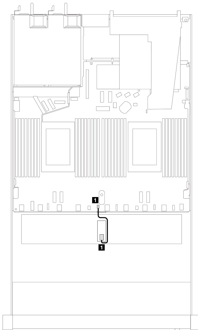
Рис. 330. Прокладка кабелей к датчику вмешательства
