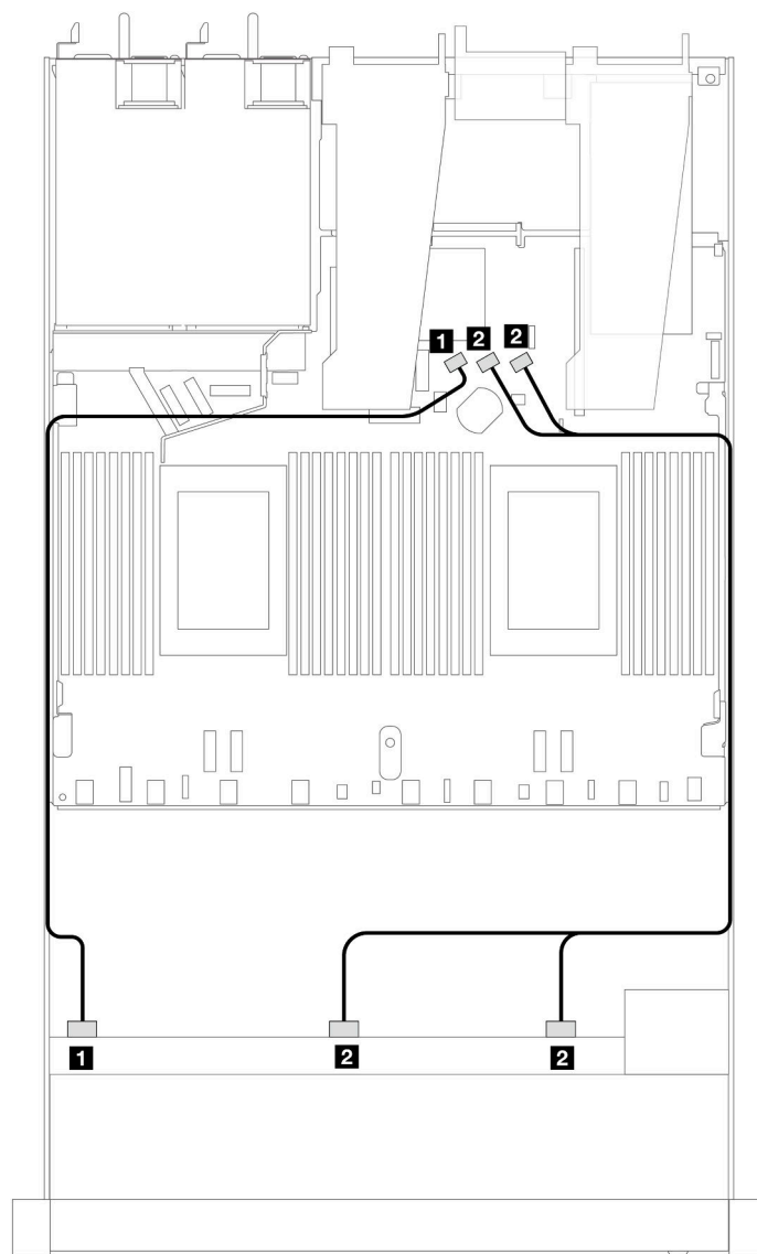
Рис. 366. Прокладка кабелей для встроенной конфигурации с 10 передними 2,5-дюймовыми дисками SAS/SATA
