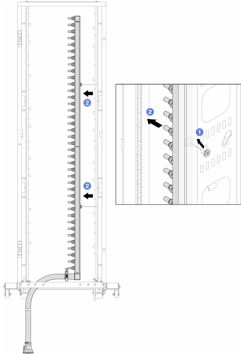
Рис. 157. Снятие коллектора
