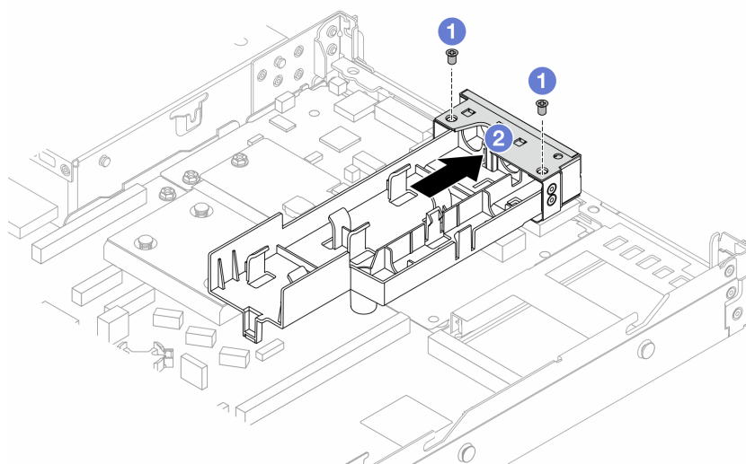
Рис. 116. Снятие кожуха держателя
