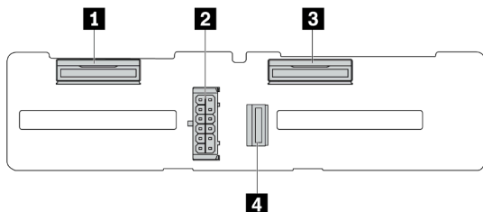
Рис. 310. Объединительная панель NVMe для четырех 2,5-дюймовых дисков
