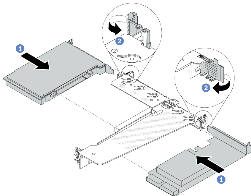
Рис. 195. Установка адаптера PCIe в блок платы-адаптера Riser LP-FH
