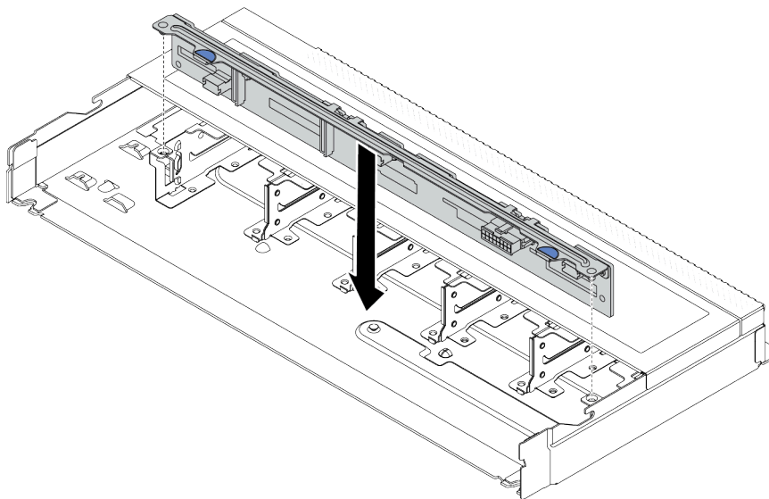
Рис. 34. Установка объединительной панели для десяти 2,5-дюймовых оперативно заменяемых дисков
