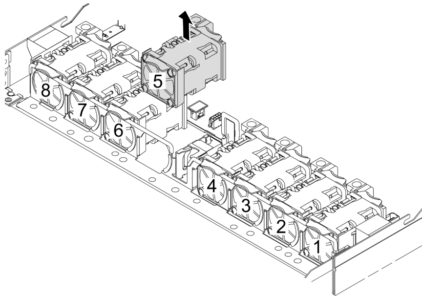
Рис. 297. Снятие вентилятора компьютера
