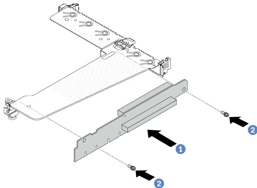
Рис. 274. Установка платы-адаптера Riser
