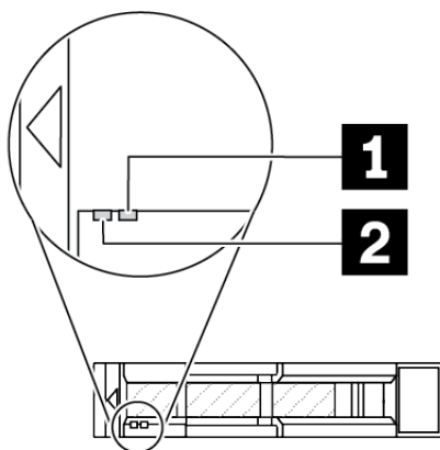
Рис. 502. Светодиодные индикаторы на жестких или твердотельных дисках
