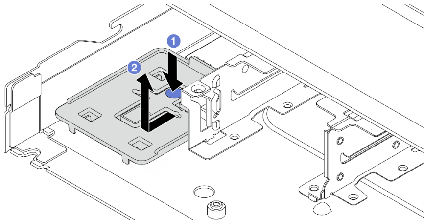
Рис. 216. Снятие лотка
