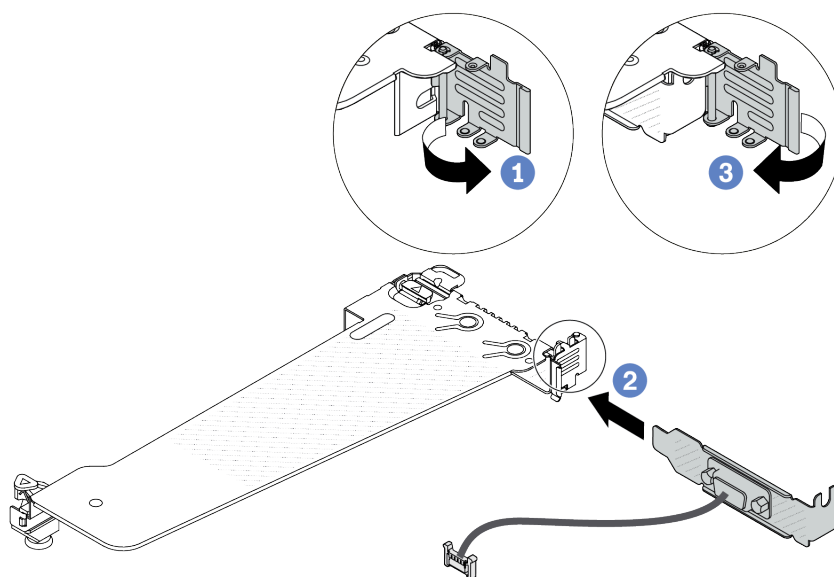
Рис. 285. Установка модуля последовательного порта
