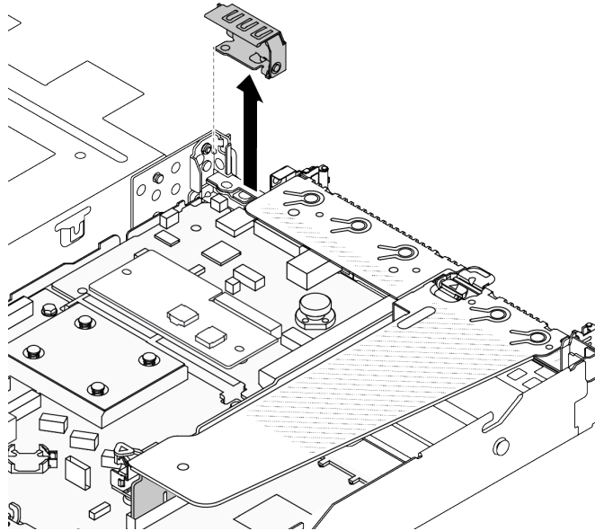
Рис. 273. Снятие скобы задней стенки
