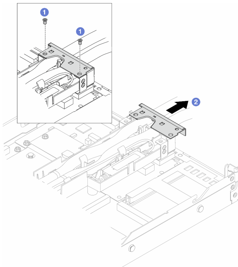
Рис. 111. Снятие кожуха держателя
