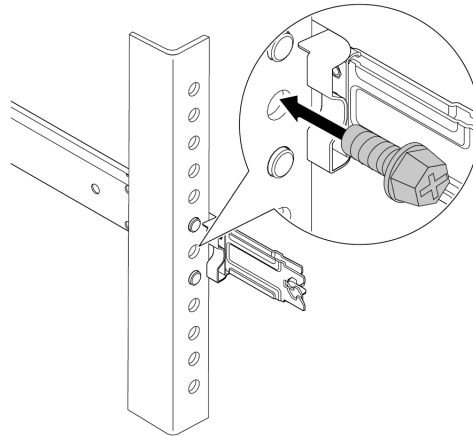
Рис. 29. Фиксация сервера на задней стороне стойки
