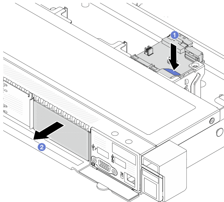
Рис. 190. Снятие отсека M.2
