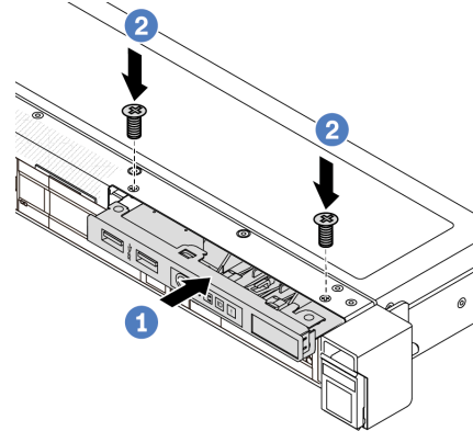
Рис. 77. Установка переднего модуля ввода-вывода в 3,5-дюймовую раму
