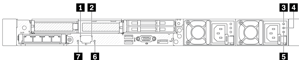
Рис. 506. Обзор светодиодных индикаторов на задней панели
