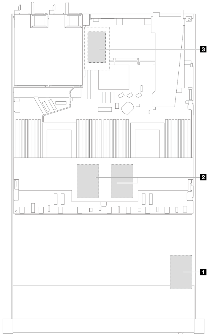
Рис. 332. Модули питания флэш-памяти RAID на раме
