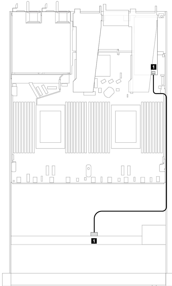
Рис. 379. Прокладка кабелей для конфигурации с четырьмя передними отсеками для 3,5-дюймовых дисков SAS/SATA и адаптером RAID 8i SFF
