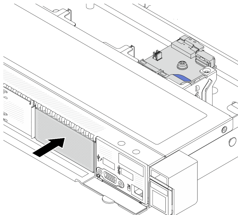
Рис. 193. Установка отсека M.2
