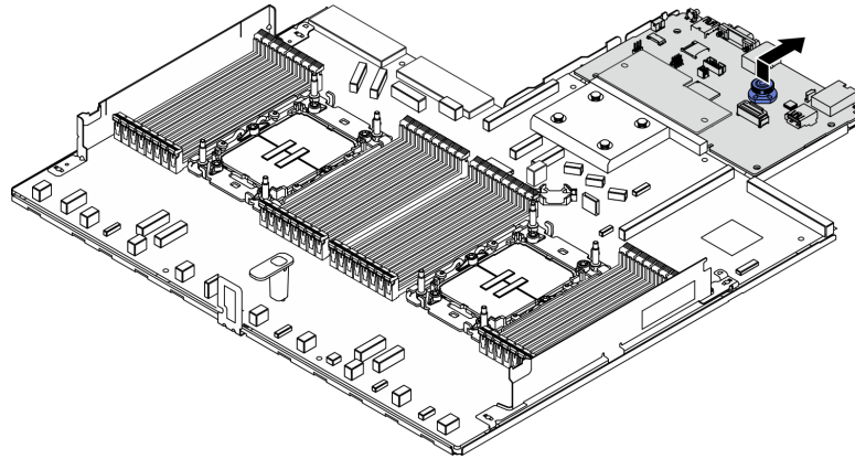
Рис. 513. Разборка платы ввода-вывода
