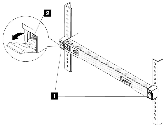
Рис. 22. Отсоединение сервера от стойки
