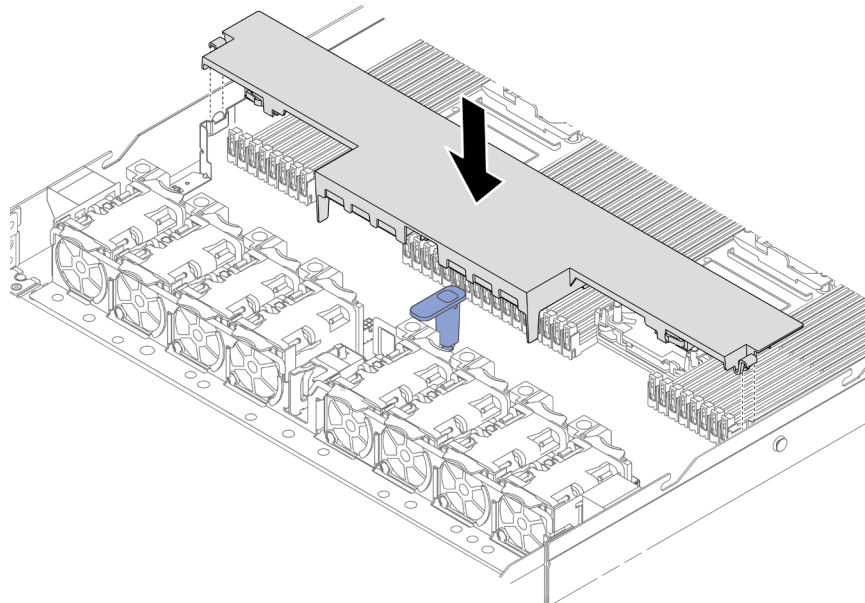
Рис. 32. Установка дефлектора
