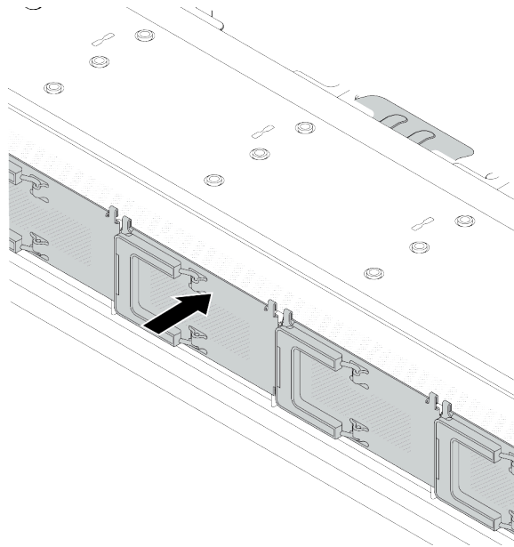
Рис. 102. Установка кожуха отсека для дисков EDSFF
