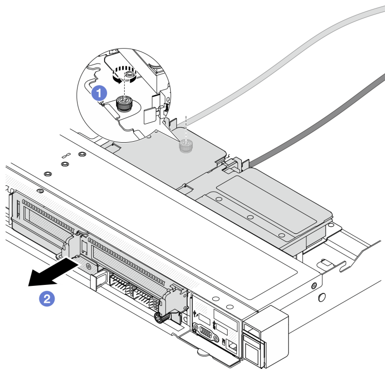
Рис. 58. Снятие переднего отсека платы-адаптера Riser
