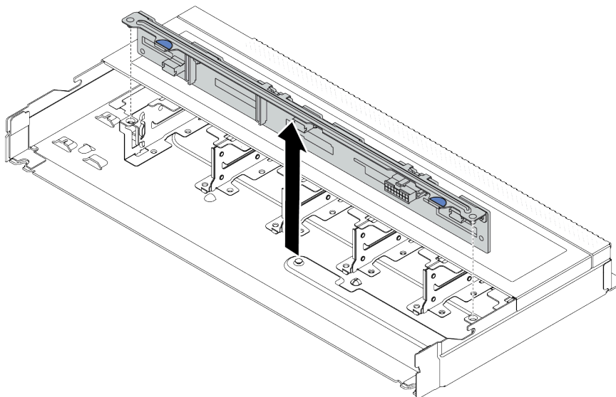
Рис. 33. Снятие объединительной панели для десяти 2,5-дюймовых оперативно заменяемых дисков
