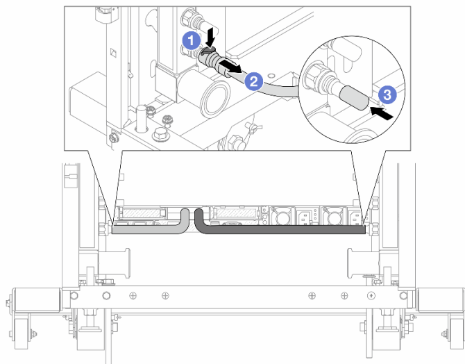
Рис. 156. Отсоединение быстроразъемного соединителя
