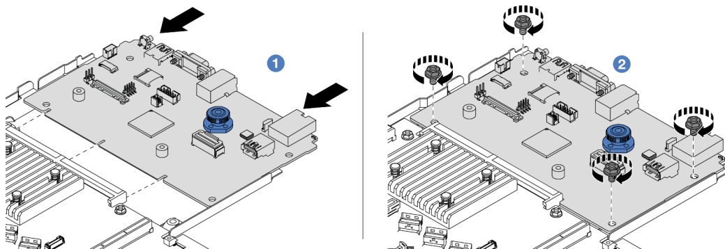
Рис. 291. Установка системной платы ввода-вывода
