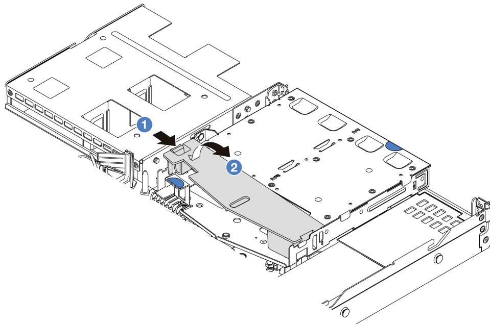
Рис. 224. Снятие дефлектора
