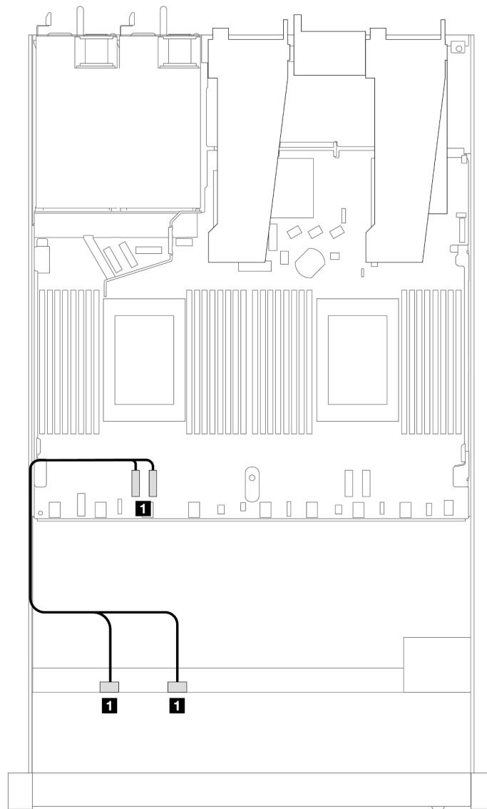
Рис. 425. Прокладка кабелей для встроенной конфигурации с 4 передними отсеками для 2,5-дюймовых дисков NVMe и двумя процессорами
