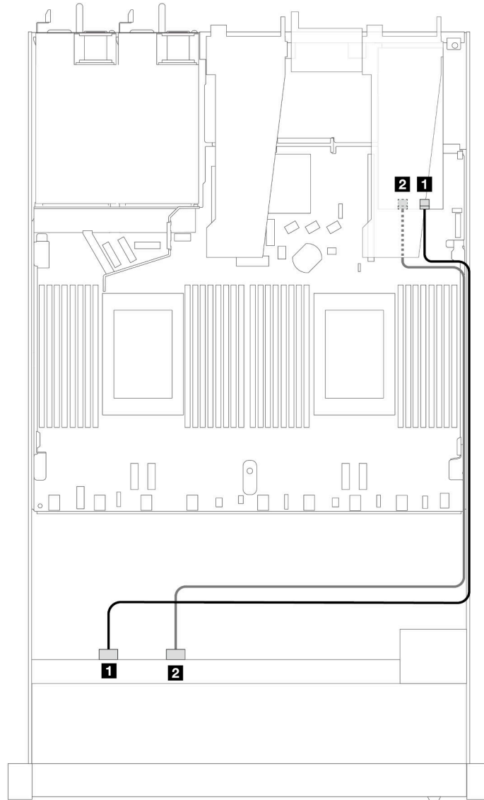
Рис. 386. Прокладка кабелей для 4 передних отсеков для 2,5-дюймовых дисков NVMe и адаптера ретаймера (Gen 4) с одним процессором
