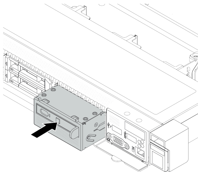
Рис. 82. Установка блока панели диагностики
