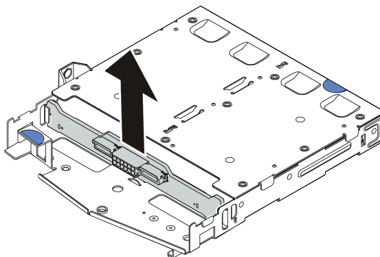
Рис. 40. Снятие задней объединительной панели для 2,5-дюймовых дисков
