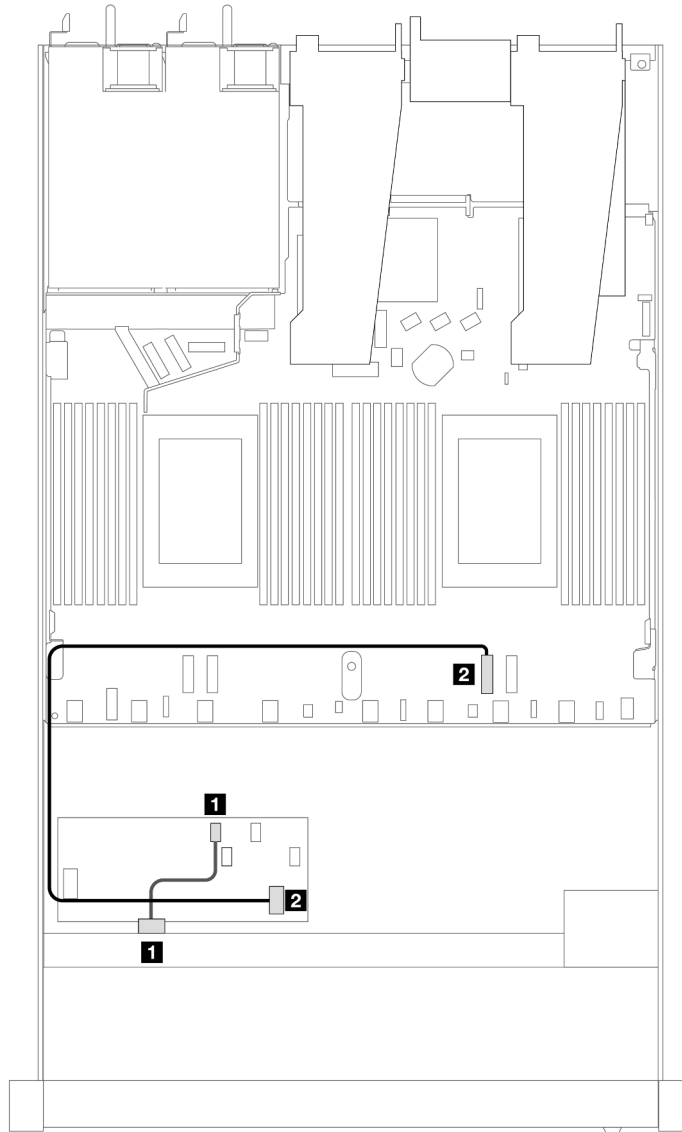
Рис. 384. Прокладка кабелей для 4 передних отсеков для 2,5-дюймовых дисков SAS/SATA с установленным адаптером RAID 8i CFF
