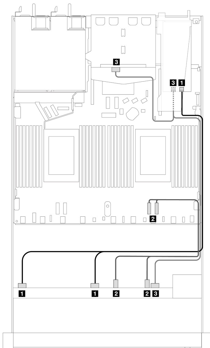
Рис. 402. Прокладка кабелей для шести передних дисков SAS/SATA, четырех отсеков для передних дисков AnyBay и адаптера RAID 16i SFF (Gen 4) с двумя установленными задними 2,5-дюймовыми дисками SAS/SATA
