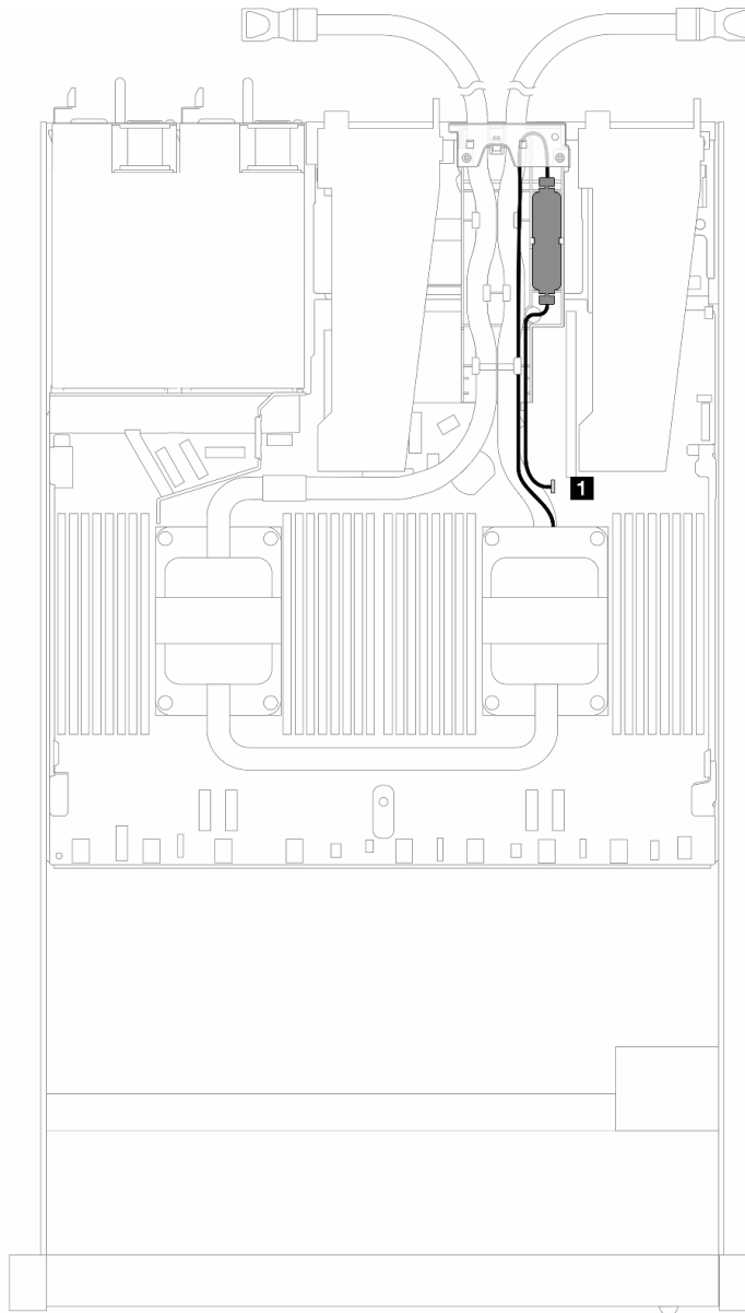
Рис. 349. Прокладка кабелей модуля непосредственного водяного охлаждения
