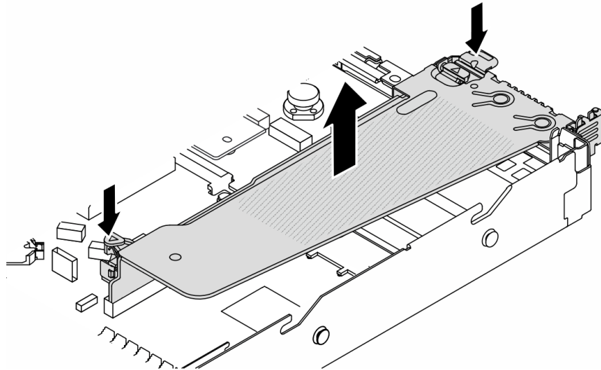
Рис. 281. Снятие скобы платы-адаптера Riser
