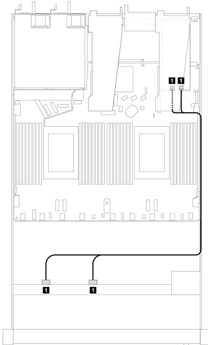
Рис. 363. Прокладка кабелей для 8 передних отсеков для 2,5-дюймовых дисков SAS/SATA и адаптера RAID 8i или 16i SFF (Gen 3)
