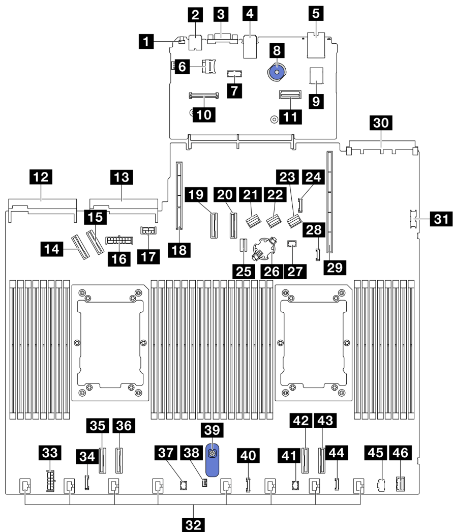
Рис. 15. Разъемы блока материнской платы
