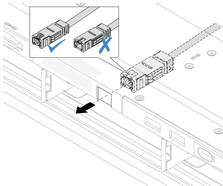
Рис. 90. Установка внешнего кабеля LCD
