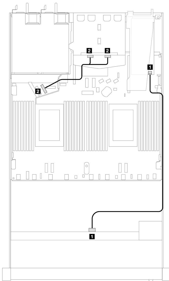
Рис. 419. Прокладка кабелей для конфигурации с четырьмя передними отсеками для 3,5-дюймовых дисков SAS/SATA, адаптером RAID 8i SFF и двумя задними 2,5-дюймовыми дисками NVMe
