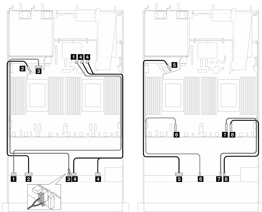
Рис. 489. Прокладка кабелей для встроенной конфигурации с 10 передними 2,5-дюймовыми дисками ApyBay
