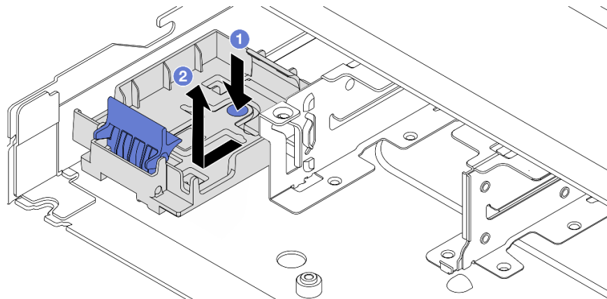
Рис. 215. Снятие держателя модуля питания флэш-памяти RAID
