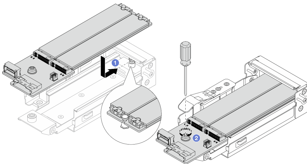
Рис. 192. Установка объединительной панели M.2
