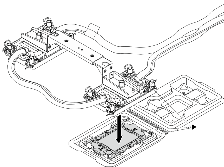
Рис. 117. Установка процессора
