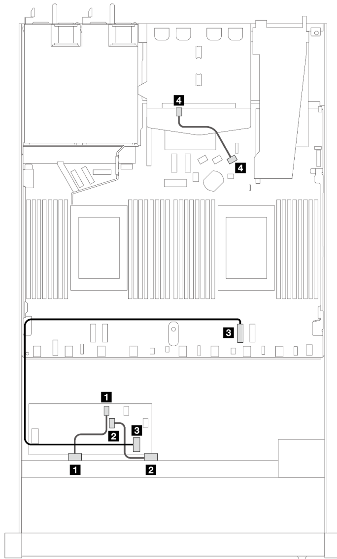
圖例 375. 配備 8i CFF RAID 配接卡 (Gen 3) (已安裝 2 x 2.5 SAS/SATA 硬碟) 之 8 x 2.5 吋前方 SAS/SATA 機槽的纜線佈線
