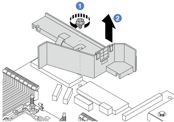
圖例 176. 卸下電源供應器空氣擋板
