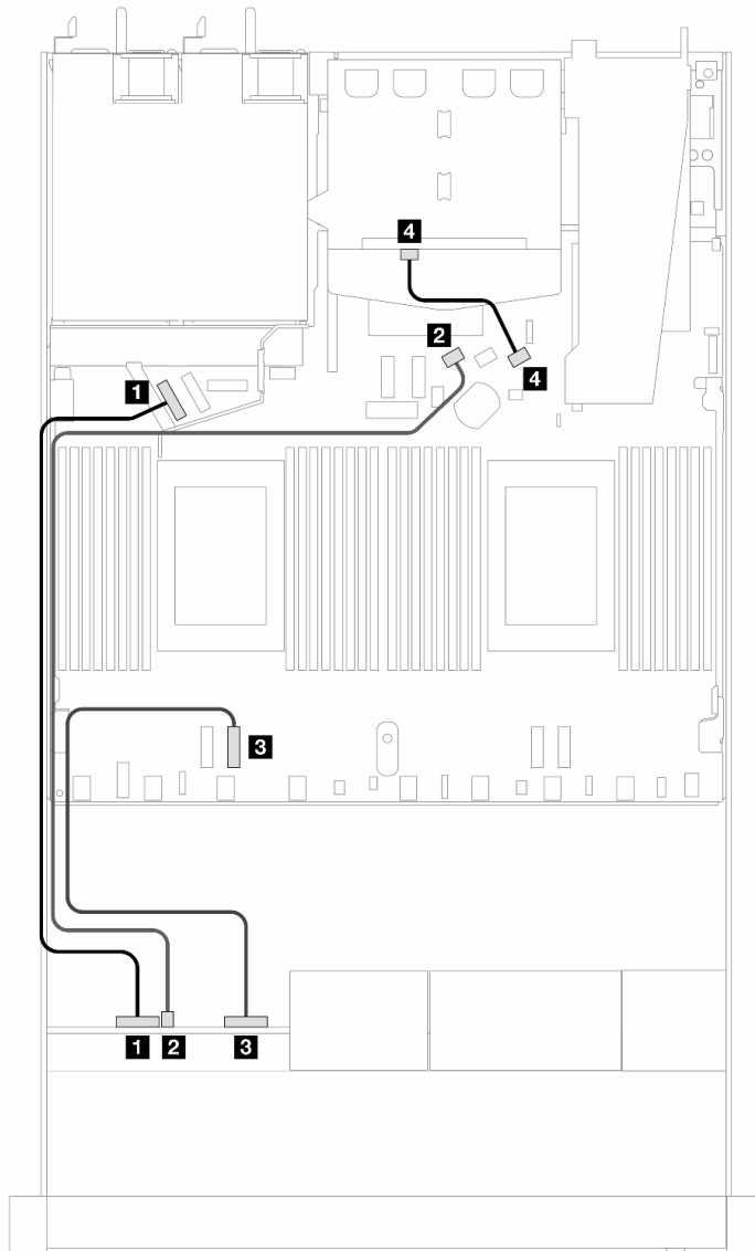
圖例 417. 4 x 2.5 吋前方 AnyBay 硬碟和 2 x 2.5 吋後方 SAS/SATA 硬碟機載配置的纜線佈線
