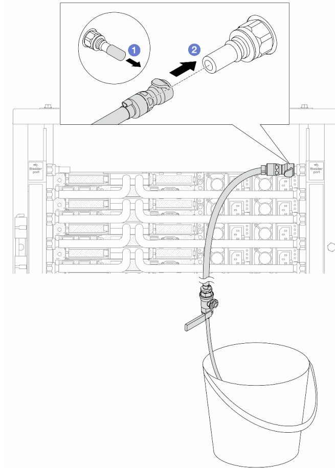
圖例 149. 在回流側安裝洩放套件
