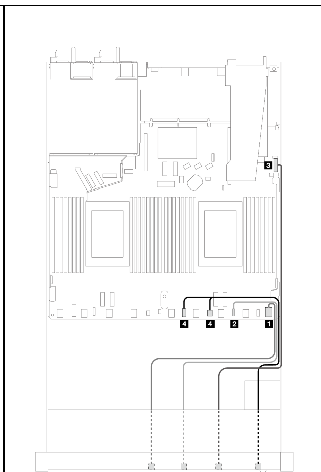
圖例 308. 3.5 吋機箱上正面 I/O 模組的纜線佈線
