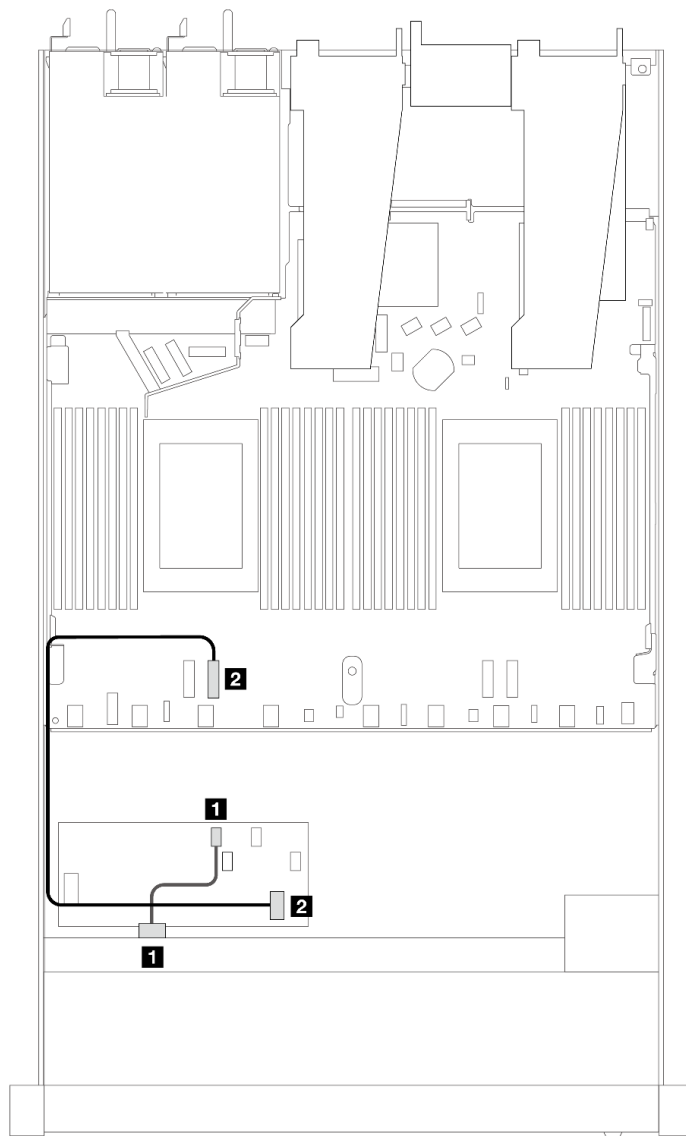
圖例 404. 已安裝 8i CFF RAID 配接卡之 4 x 2.5 吋前方 SAS/SATA 機槽的纜線佈線
