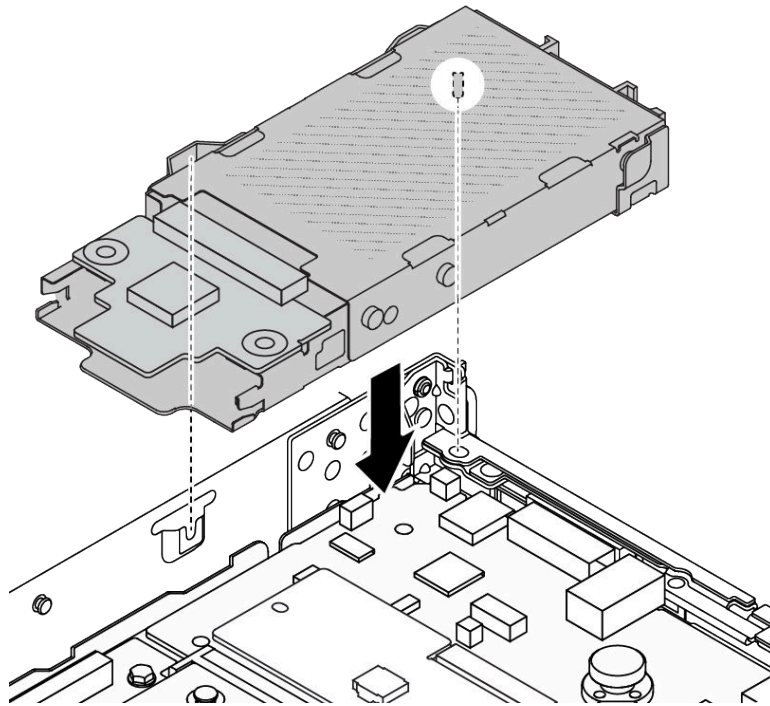
圖例 209. 安裝 7 公釐背面框架
