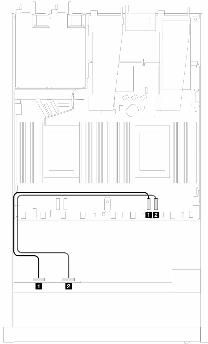
圖例 331. 用於液冷的四個 NVMe 磁碟機的機載佈線
