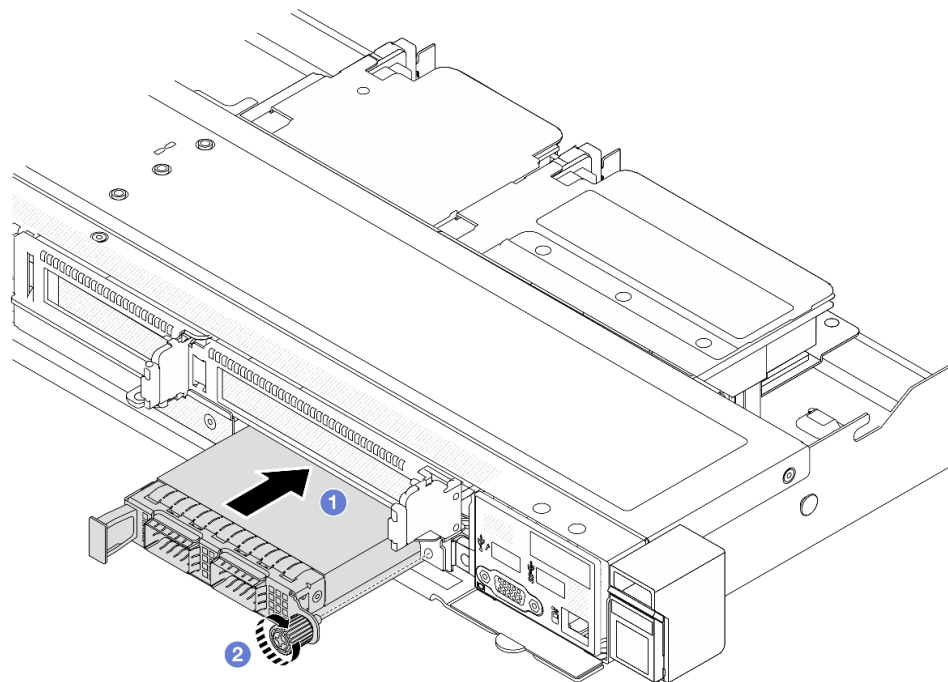
圖例 49. 安裝正面 OCP 模組
