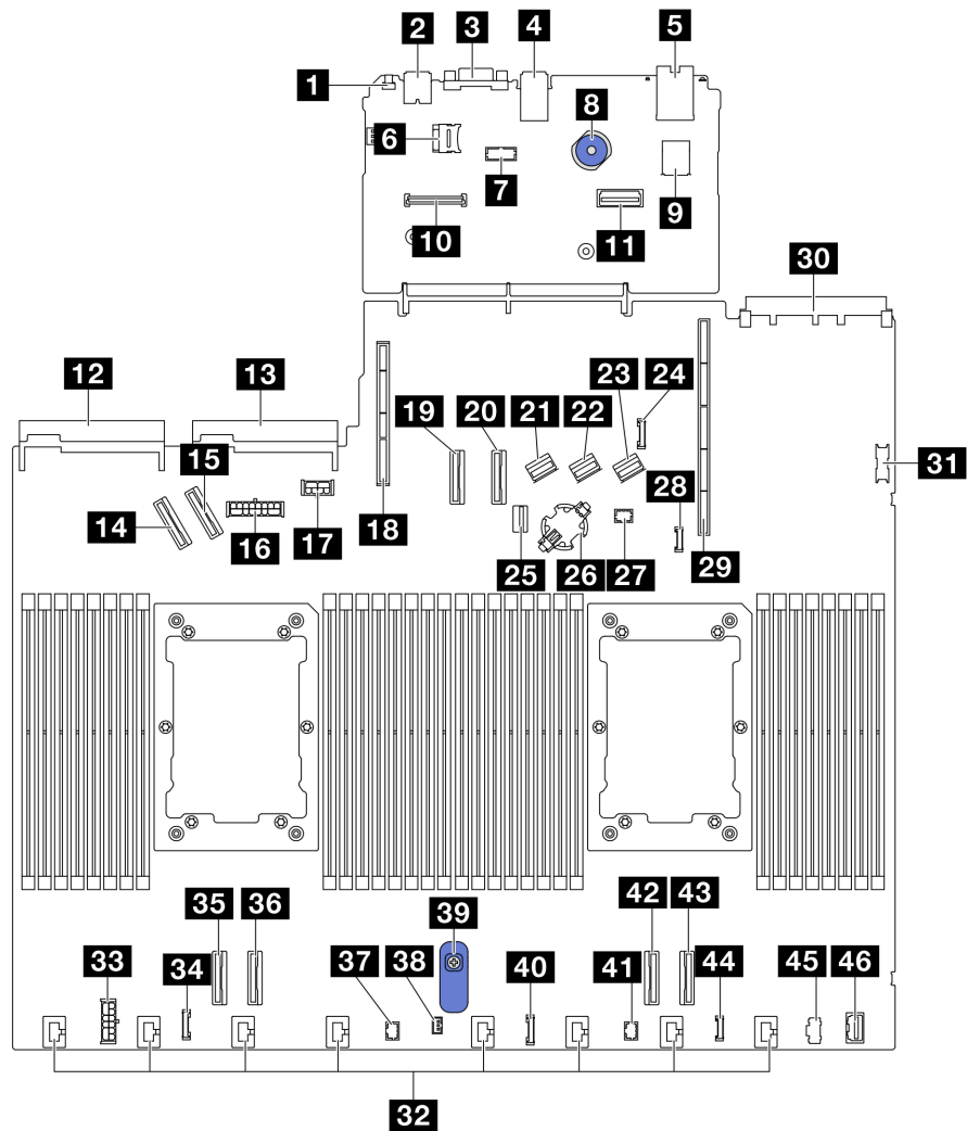
圖例 476. 主機板組件接頭
