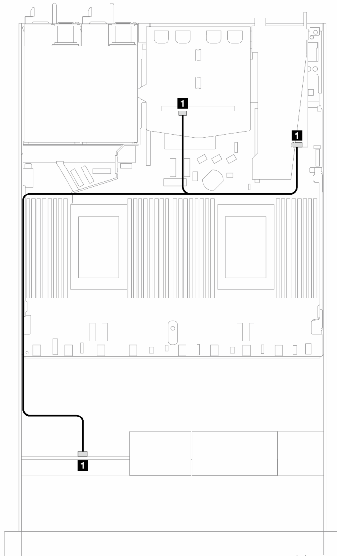
圖例 411. 包含 8i SFF RAID 配接卡 (Gen 4) 和 2 x 2.5 吋後方 SAS/SATA 硬碟的 4 x 2.5 吋前方 AnyBay 機槽的纜線佈線
