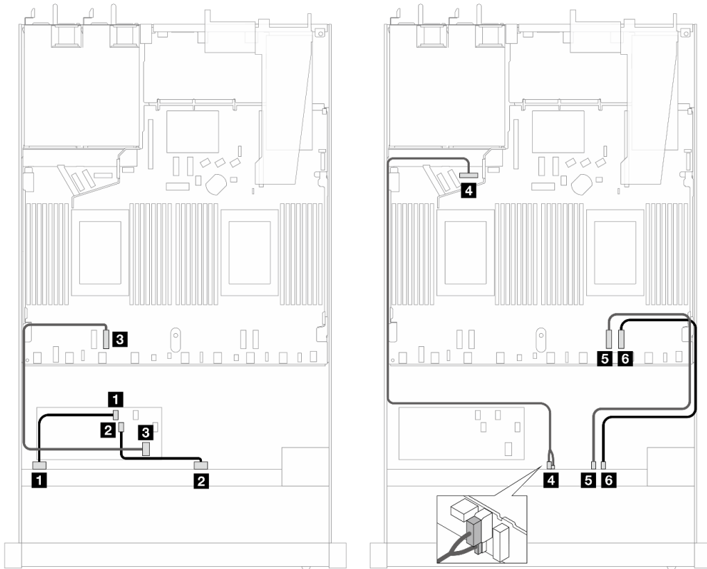
圖例 468. 包含 16i CFF HBA/RAID 配接卡 (Gen 3 或 Gen 4) 的六個 SAS/SATA 硬碟和兩個 AnyBay 硬碟和兩個 NVMe 前方機槽的纜線佈線
