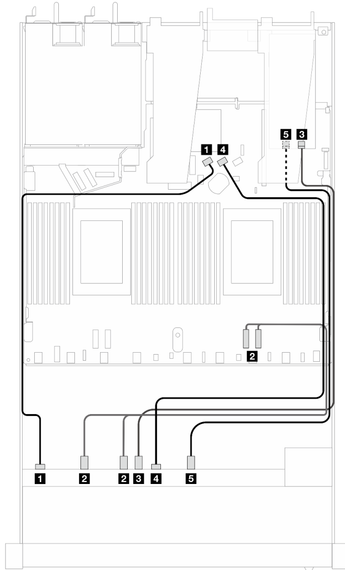
圖例 378. 八個 AnyBay 前方硬碟的纜線佈線，既可連接到板上，也可連接到 Gen 4 SFF 重定時器配接卡上
