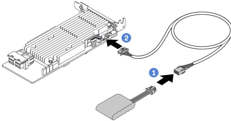
圖例 193. 快閃記憶體電源模組的電源線佈線
