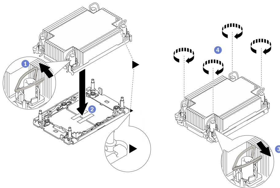
圖例 188. 安裝 PHM
