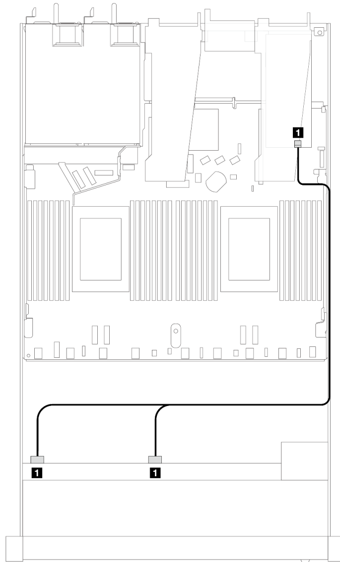
圖例 345. 包含 8i SFF RAID 配接卡 (Gen 4) 的 8 x 2.5 吋前方 U.3 硬碟纜線佈線
