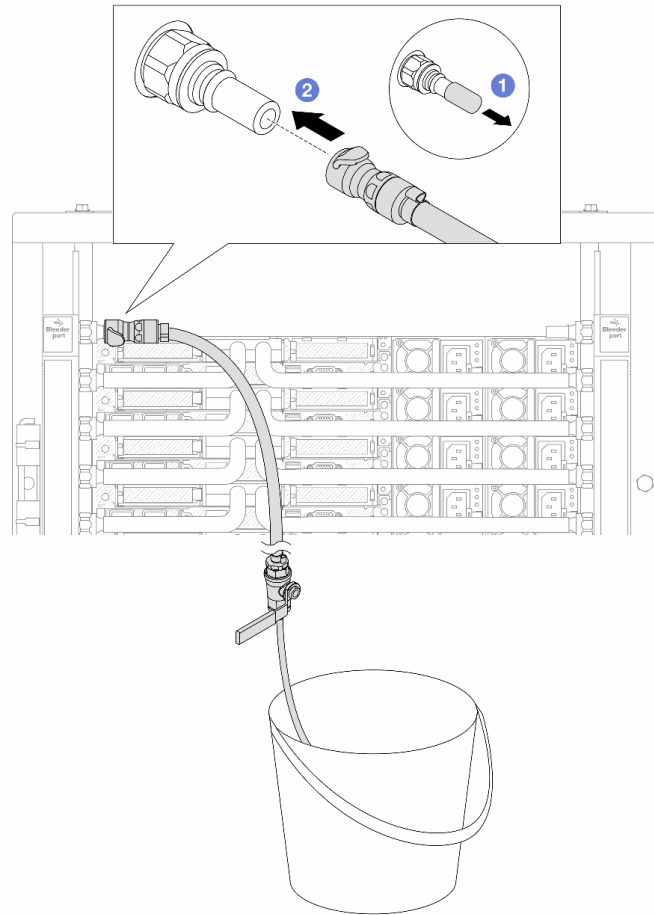
圖例 146. 安裝供應側的洩放套件
