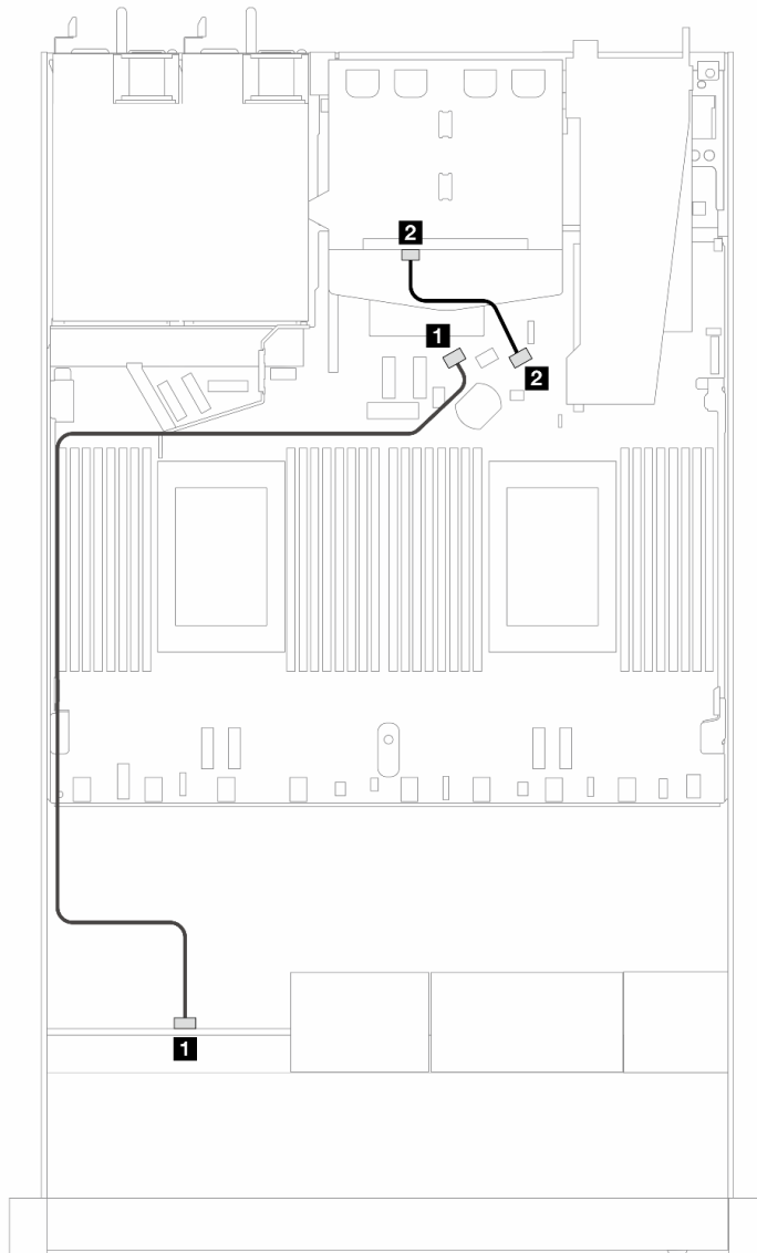
圖例 408. 4 x 2.5 吋前方 SAS/SATA 硬碟和 2 x 2.5 吋後方 SAS/SATA 硬碟機載配置的纜線佈線
