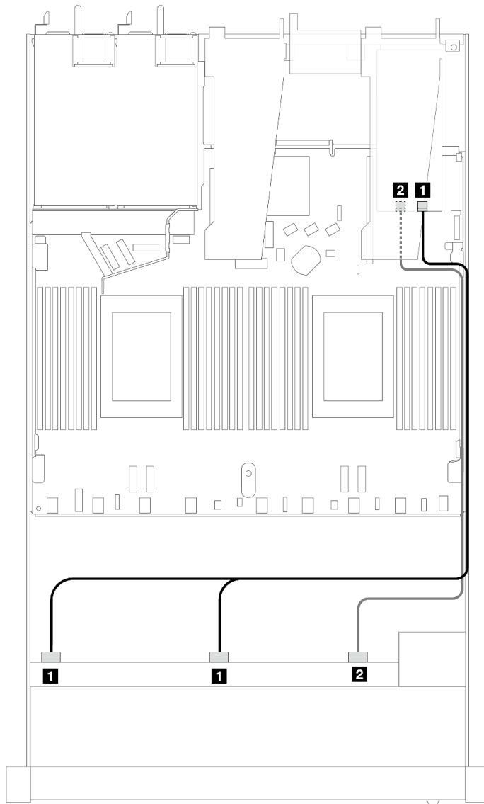
圖例 389. 包含 16i SFF RAID 配接卡 (Gen 4) 的 10 個前方 SAS/SATA 硬碟的纜線佈線
