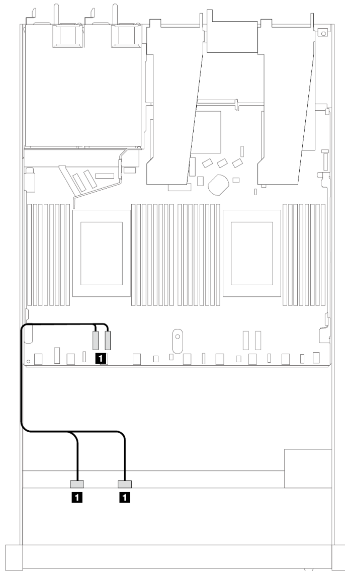
圖例 405. 包含兩個處理器的 4 x 2.5 吋前方 NVMe 機槽機載配置的纜線佈線
