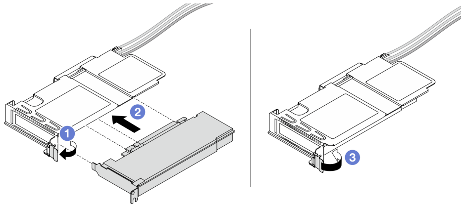
圖例 46. 安裝 PCIe 配接卡
