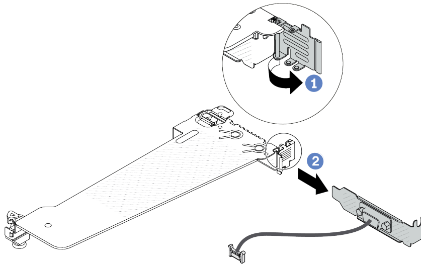
圖例 262. 卸下擴充卡托架
