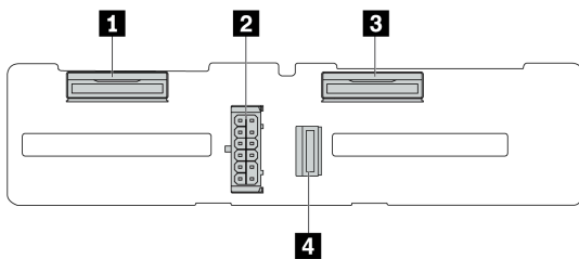
圖例 290. 4 x 2.5 吋 NVMe 背板
