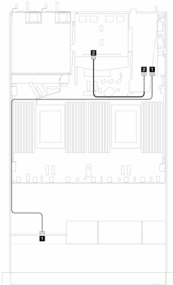
圖例 410. 包含 8i SFF RAID 配接卡 (Gen 3) 和 2 x 2.5 吋後方 SAS/SATA 硬碟的 4 x 2.5 吋前方 AnyBay 機槽的纜線佈線
