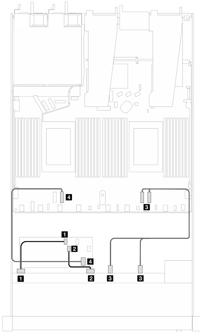
圖例 444. 包含 8i 或 16i CFF RAID 配接卡 ( Gen 3 或 Gen 4 ) 的 6 個 SAS/SATA 硬碟和 2 個 AnyBay 硬碟和 2 個 NVMe 前方機槽的纜線佈線
