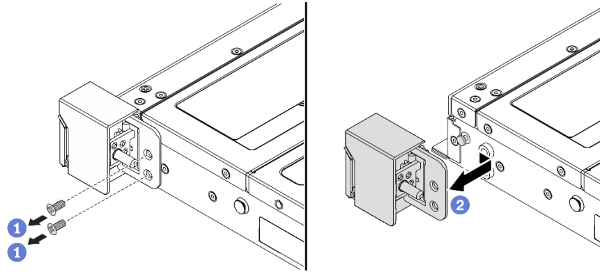
圖例 190. 機架門鎖拆卸
