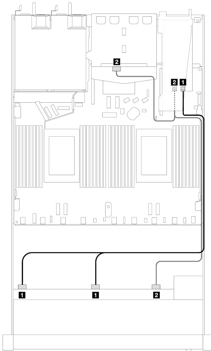
圖例 447. 安裝 2 x 2.5 後方 SAS/SATA 硬碟之 10 個前方 SAS/SATA 機槽和 16i SFF RAID 配接卡 (Gen 4) 的纜線佈線
