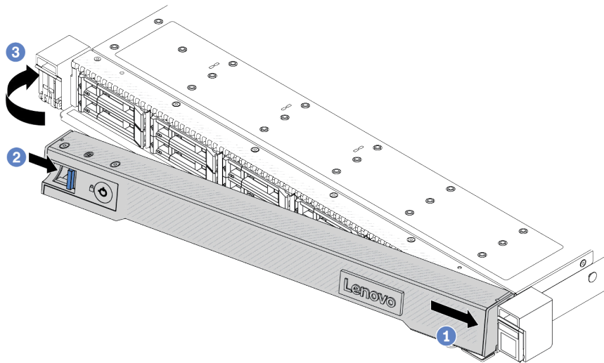
圖例 259. 安裝安全擋板
