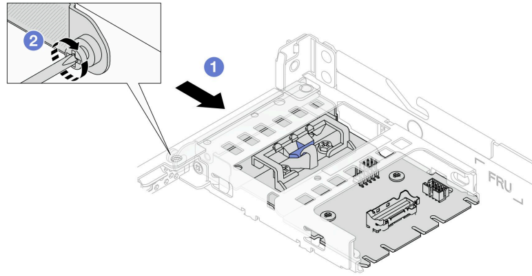
圖例 53. 安裝背面 OCP 轉插卡
