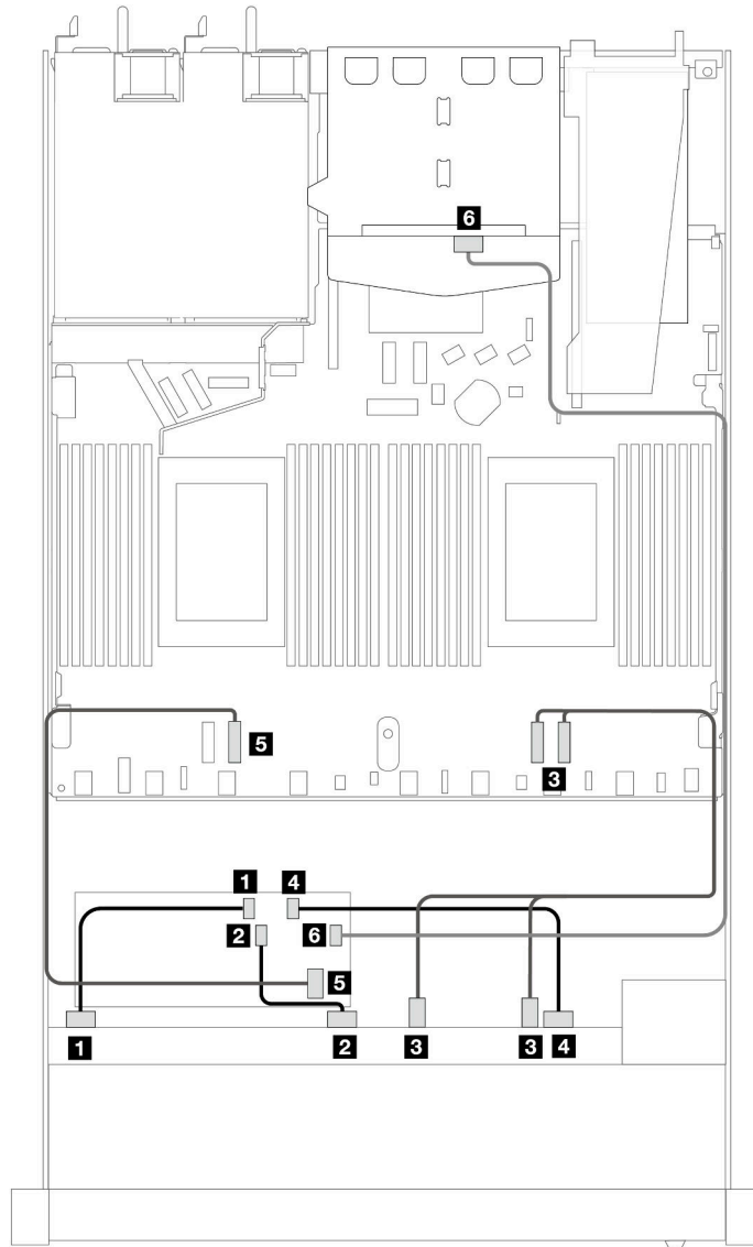
圖例 440. 6 個前方 SAS/SATA 硬碟和 4 個前方 AnyBay 機槽以及 16i CFF RAID 配接卡 ( Gen 3 或 Gen 4 ) ( 已安裝 2 x 2.5 後方 SAS/SATA 硬碟 ) 的纜線佈線
