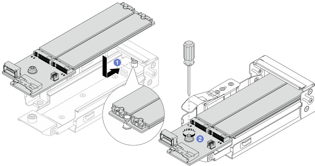
圖例 172. M.2 背板安裝
