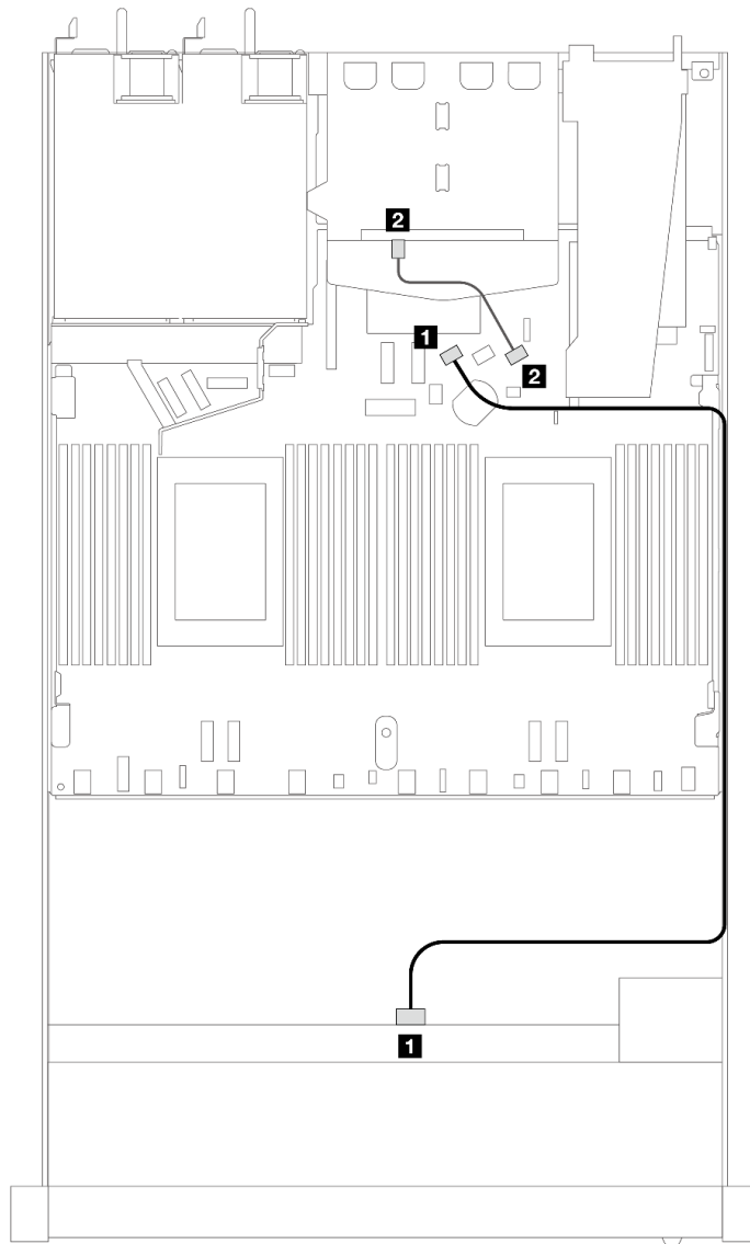
圖例 358. 配備 2 x 2.5 後方 SAS/SATA 硬碟之 4 x 3.5 吋前方 SAS/SATA 機槽機載配置的纜線佈線
