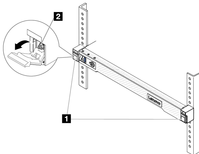
圖例 10. 將伺服器固定到機架正面
