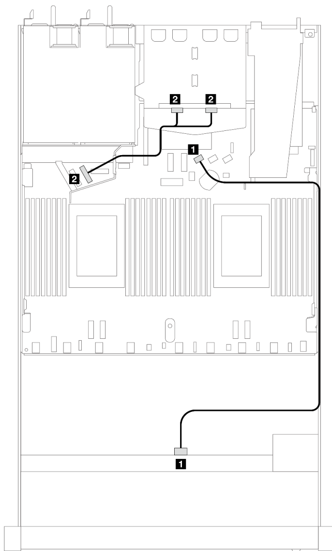
圖例 396. 配備 2 x 2.5 後方 NVMe 硬碟之 4 x 3.5 吋前方 SAS/SATA 硬碟機載配置的纜線佈線
