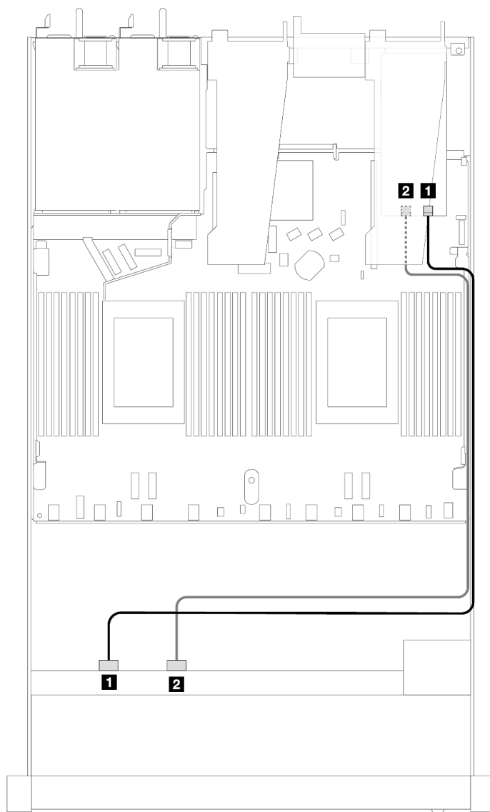
圖例 366. 包含一個處理器的 4 x 2.5 吋前方 NVMe 機槽和重定時器配接卡 (Gen 4) 的纜線佈線
