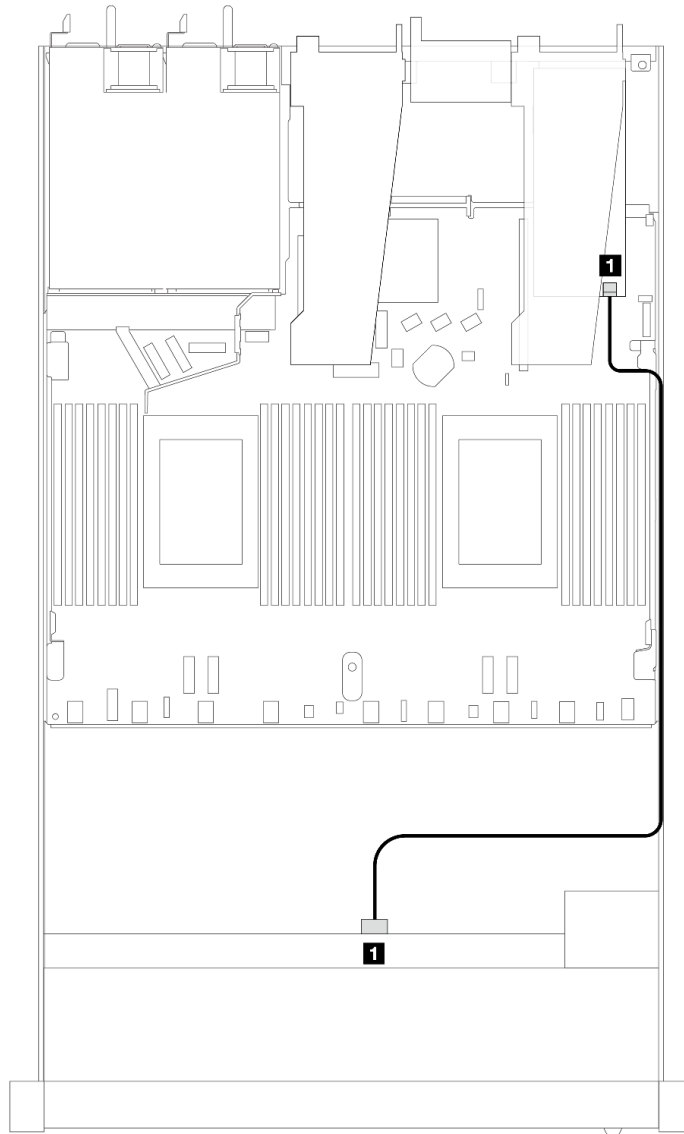
圖例 406. 包含 8i SFF RAID 配接卡 (Gen 4) 的 4 x 2.5 吋前方 U.3 硬碟纜線佈線
