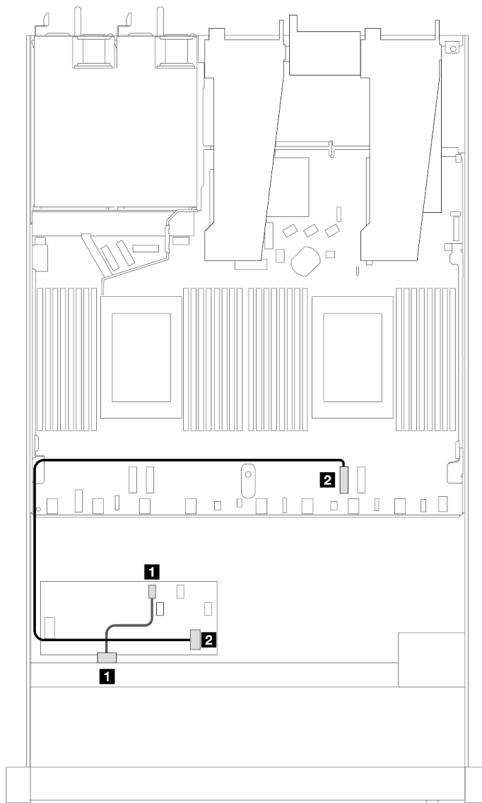
圖例 364. 已安裝 8i CFF RAID 配接卡之 4 x 2.5 吋前方 SAS/SATA 機槽的纜線佈線
