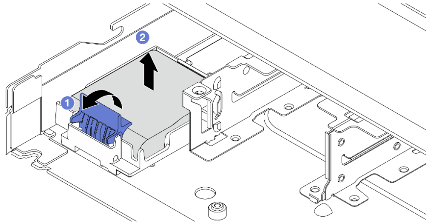
圖例 194. 卸下機箱上的 RAID 快閃記憶體電源模組
