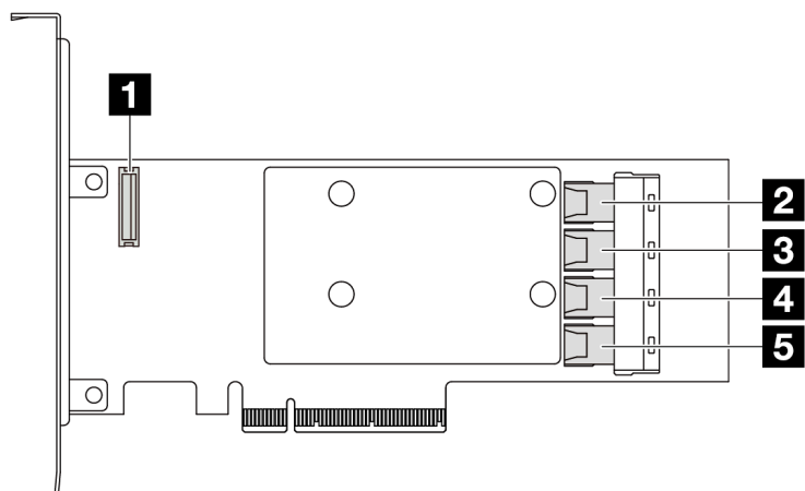
圖例 297. Gen 3 16i SFF RAID/HBA 配接卡 ( 四個埠接頭 )
