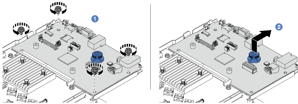
圖例 270. 卸下系統 I/O 板
