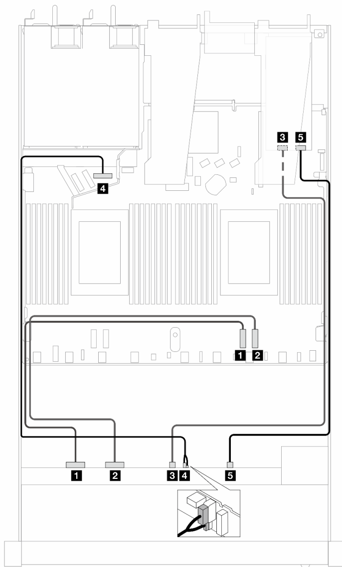
圖例 344. 八個 U.2 前方硬碟的纜線佈線，既可連接到板上，也可連接到 Gen 5 SFF 重定時器配接卡上
