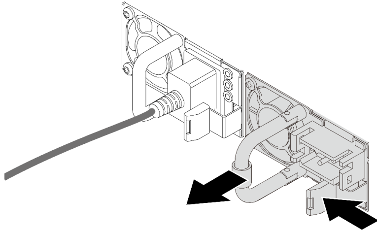
圖例 84. 卸下熱抽換電源供應器
