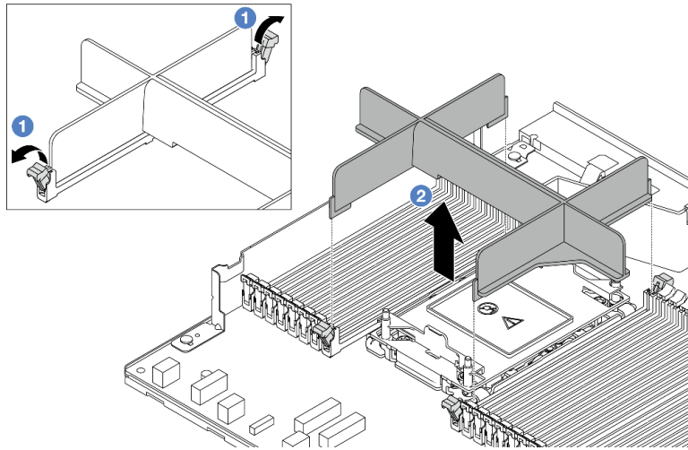
圖例 187. 卸下 PHM 填充板
