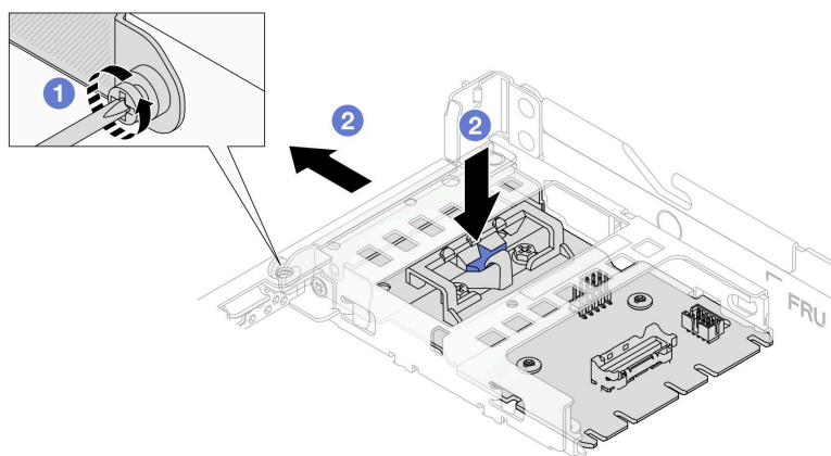
圖例 52. 卸下背面 OCP 轉插卡
