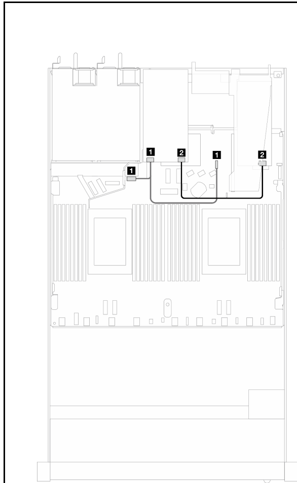
圖例 323. 7 公釐背板到 Gen 3 SFF RAID 配接卡
