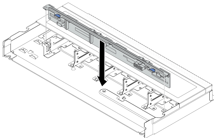
圖例 14. 安裝十個 2.5 吋熱抽換硬碟的背板
