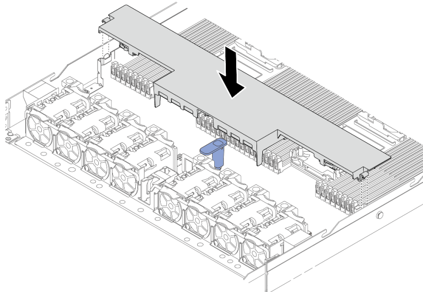
圖例 12. 安裝空氣擋板
