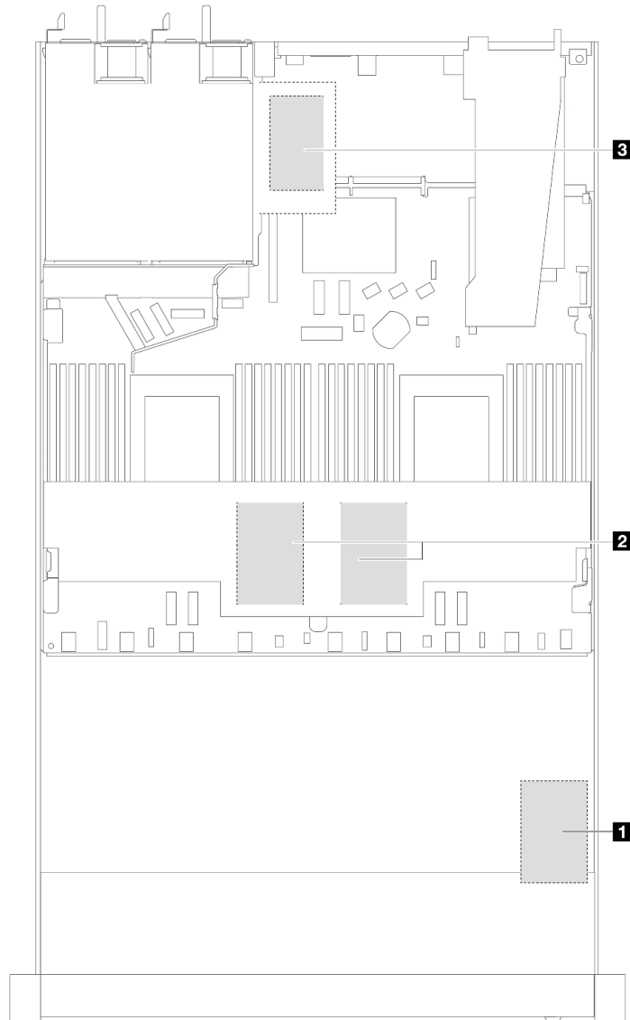
圖例 312. 機箱中的 RAID 快閃記憶體電源模組
