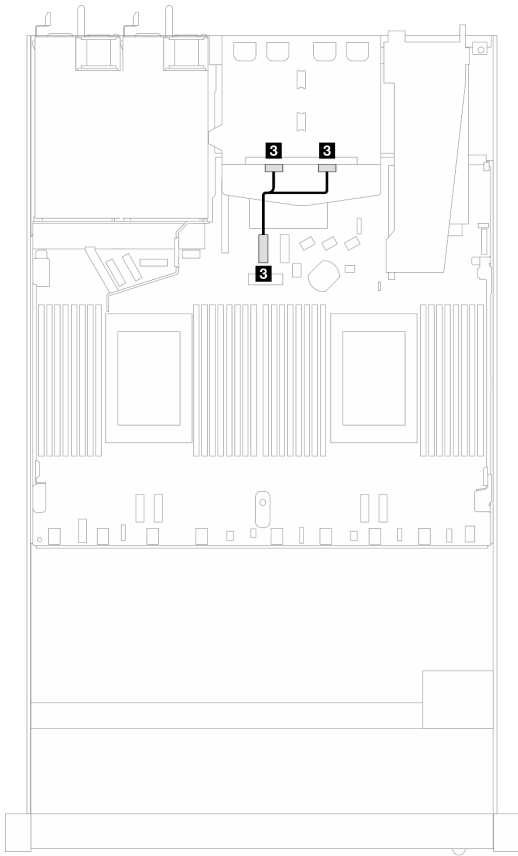
圖例 327. 後方 NVMe 背板信號線與處理器板之間的映射
