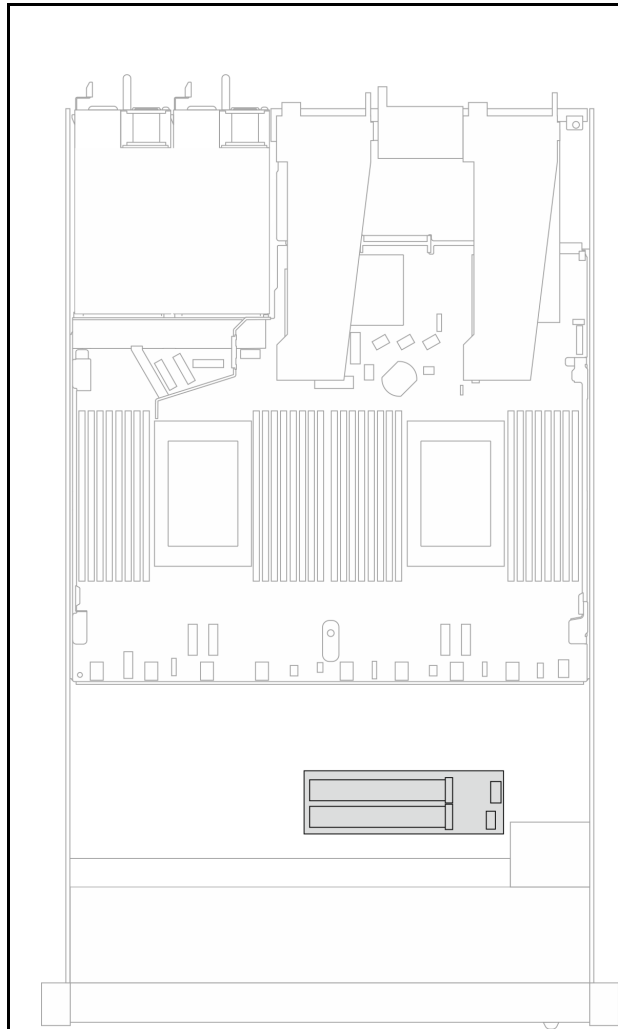
圖例 318. 2.5/3.5 吋硬碟機箱中的 M.2 硬碟組件
