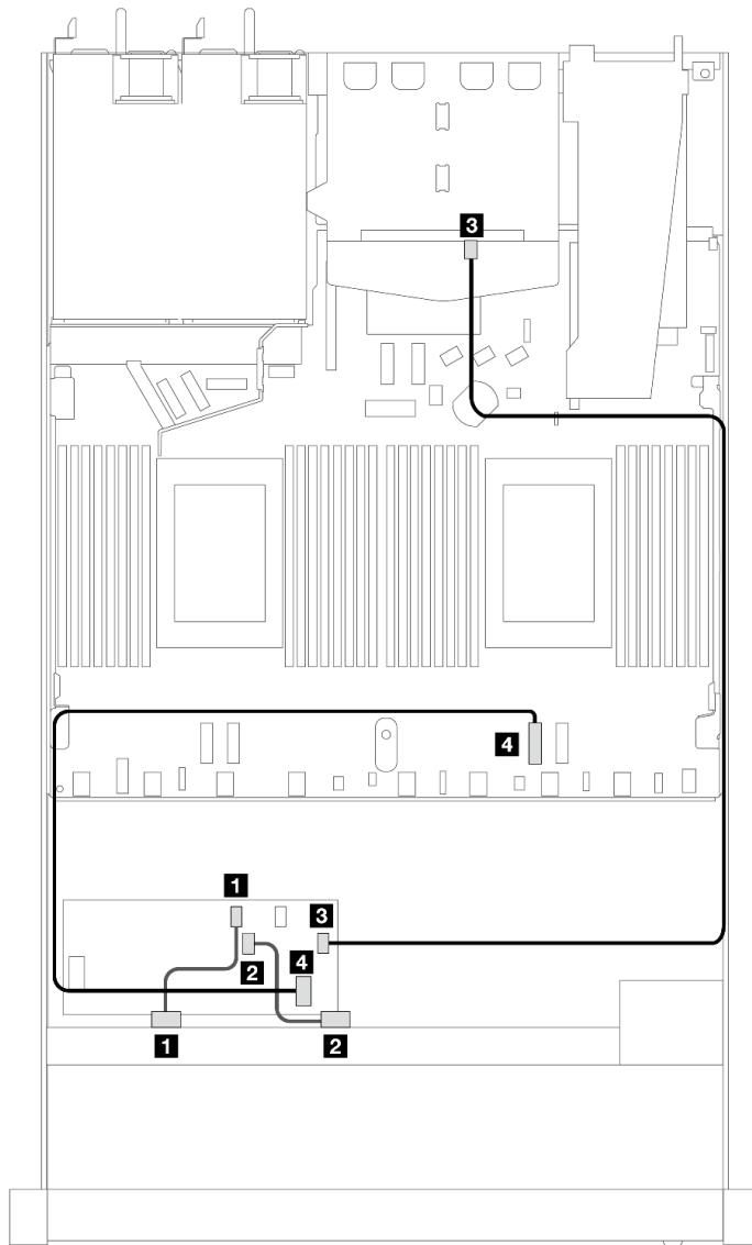
圖例 376. 配備 16i CFF RAID 配接卡 ( Gen 3 或 Gen 4 ) ( 已安裝 2 x 2.5 SAS/SATA 硬碟 ) 之 8 x 2.5 吋前方 SAS/SATA 機槽的纜線佈線
