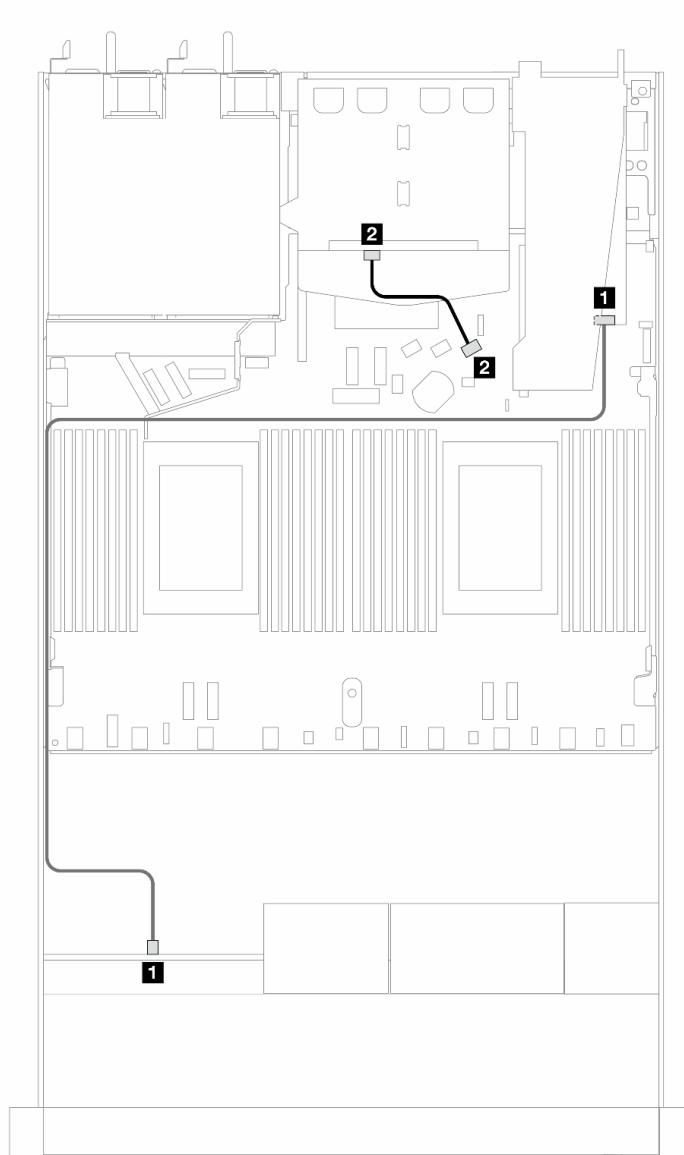
圖例 422. 包含 8i SFF RAID 配接卡 ( Gen 4 三態 ) 和 2 x 2.5 吋後方 SAS/SATA 硬碟的 4 x 2.5 吋前方 AnyBay 機槽的纜線佈線
