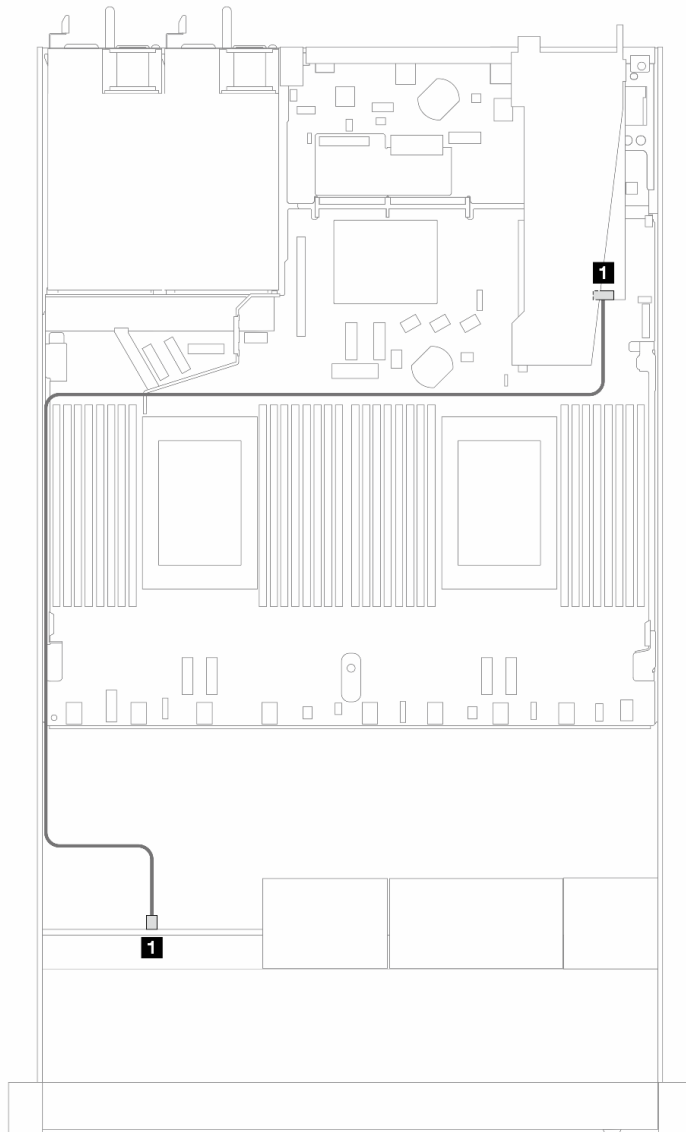
圖例 421. 包含 8i SFF RAID 配接卡 ( Gen 4 三態 ) 的 4 x 2.5 吋前方 AnyBay 機槽的纜線佈線
