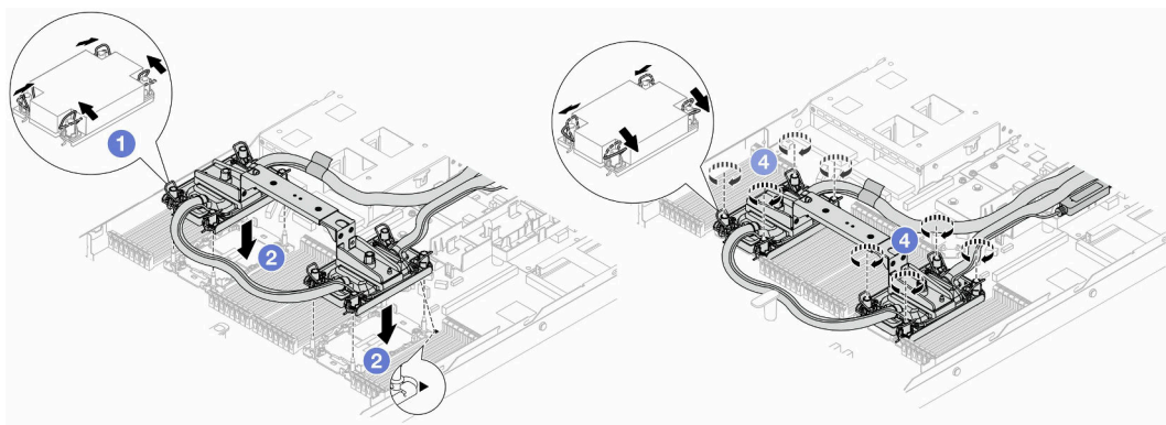
圖例 99. 安裝 DWCM
