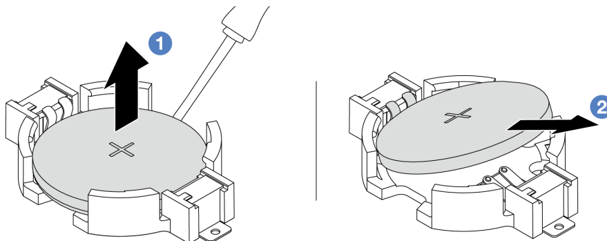
圖例 28. 卸下 CMOS 電池
