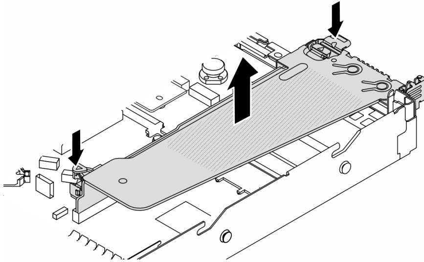
圖例 261. 卸下擴充卡托架
