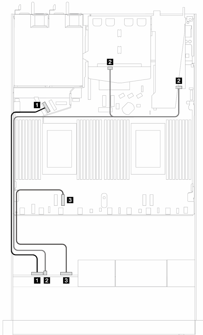
圖例 420. 包含 8i SFF RAID 配接卡 (Gen 4) 和 2 x 2.5 吋後方 SAS/SATA 硬碟的 4 x 2.5 吋前方 AnyBay 機槽的纜線佈線
