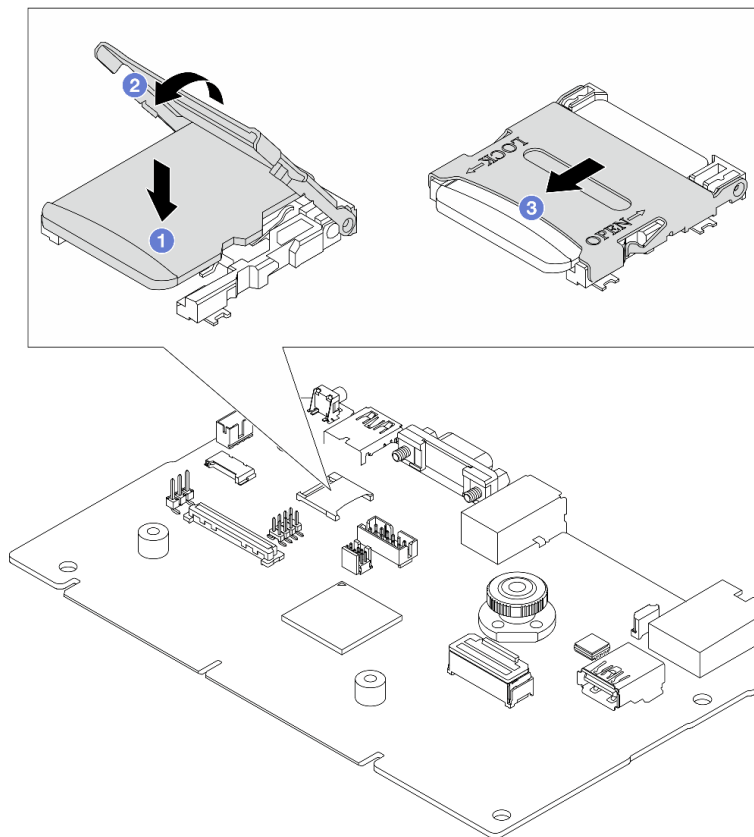
圖例 157. 安裝 MicroSD 卡
