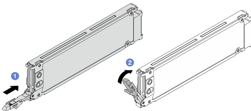
圖例 81. EDSFF 硬碟安裝
