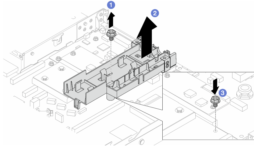
圖例 94. 卸下固定器
