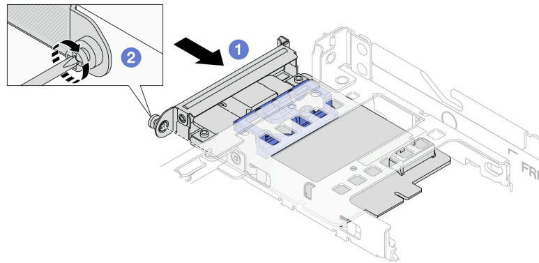
圖例 106. 安裝管理 NIC 配接卡
