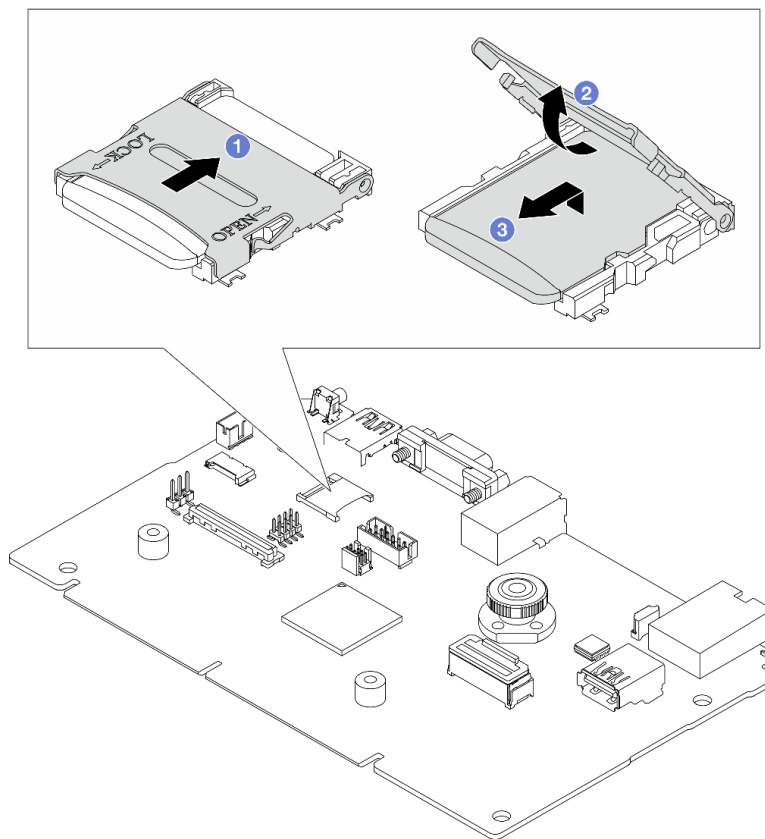
圖例 156. 卸下 MicroSD 卡
