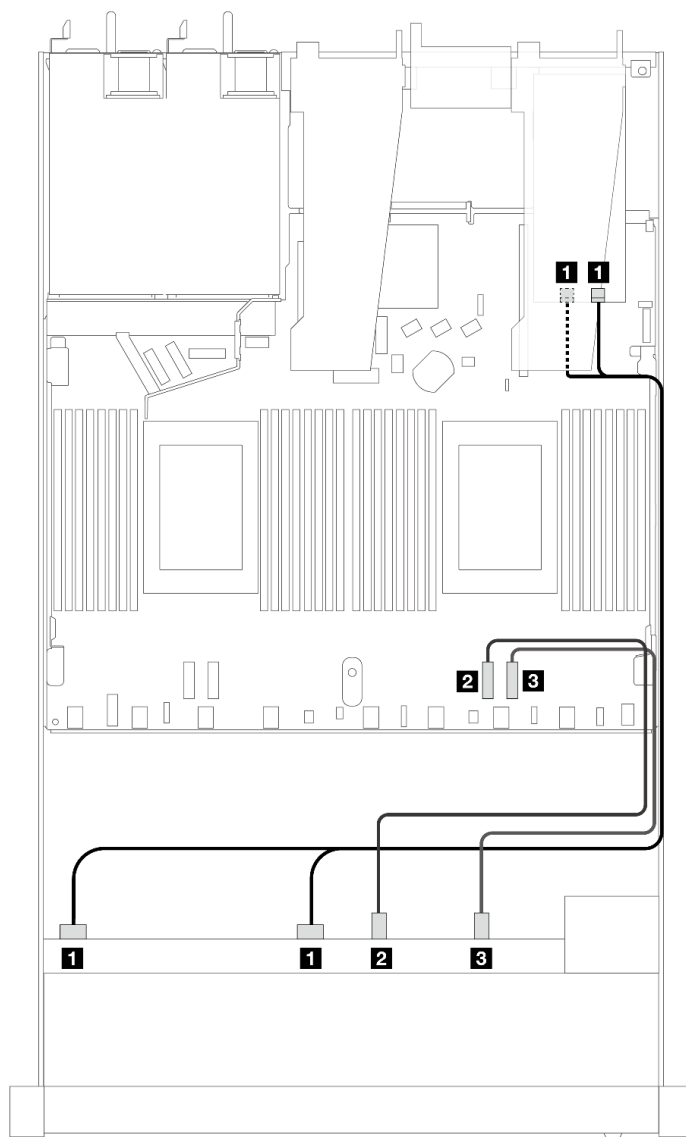
圖例 336. 包含 8i 或 16i SFF RAID 配接卡 (Gen 3) 的六個前方 SAS/SATA 硬碟和四個前方 AnyBay 機槽的纜線佈線
