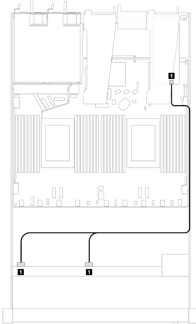
圖例 377. 包含 8i SFF RAID 配接卡 (Gen 4) 的 8 x 2.5 吋前方 U.3 硬碟纜線佈線
