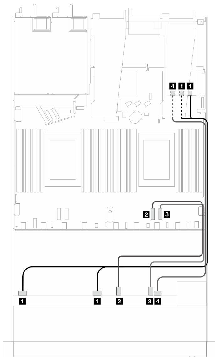
圖例 337. 包含 8i 或 16i SFF RAID 配接卡 (Gen 3) 的六個前方 SAS/SATA 硬碟和四個前方 AnyBay 機槽的纜線佈線
