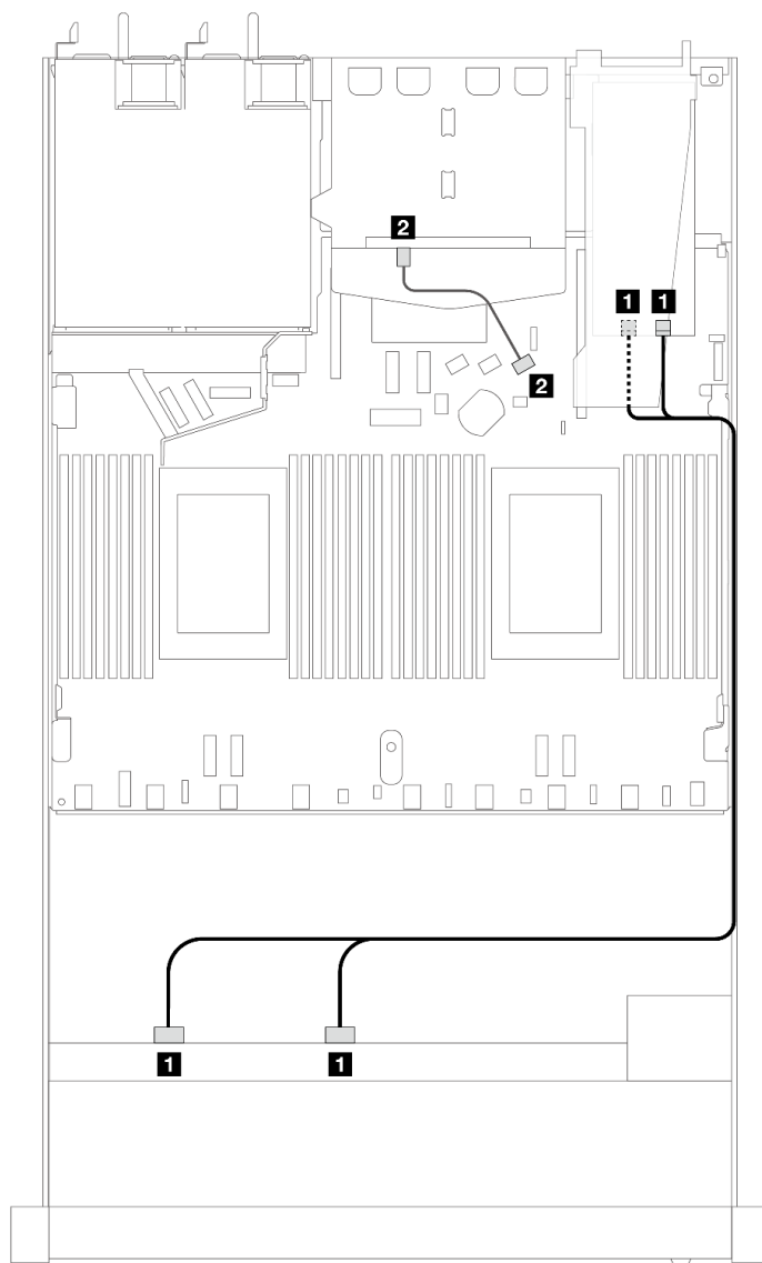
圖例 373. 配備 8i SFF RAID 配接卡 (Gen 3) (已安裝 2 x 2.5 SAS/SATA 背面硬碟) 之 8 x 2.5 吋前方 SAS/SATA 機槽的纜線佈線
