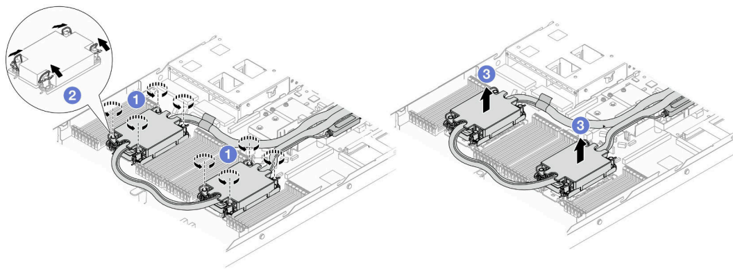
圖例 93. 卸下 DWCM
