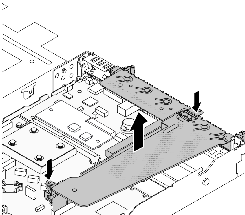
圖例 251. 卸下擴充卡組件
