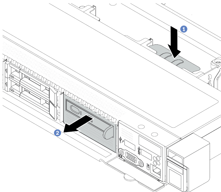
圖例 58. 卸下整合式診斷面板組件
