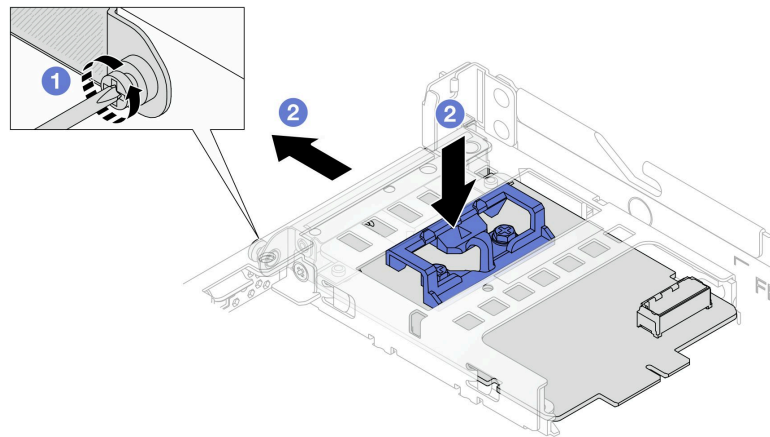
圖例 105. 卸下管理 NIC 配接卡
