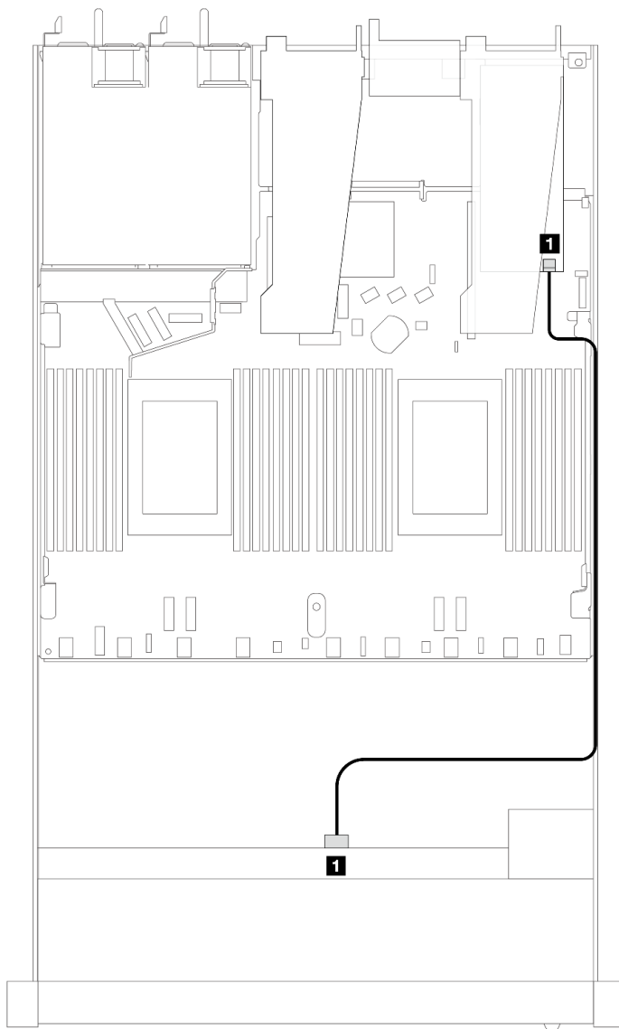
圖例 398. 包含 8i SFF RAID 配接卡的 4 x 3.5 吋前方 SAS/SATA 機槽的纜線佈線
