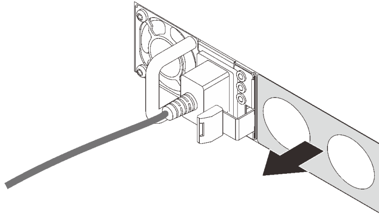
圖例 86. 卸下熱抽換電源供應器填充板
