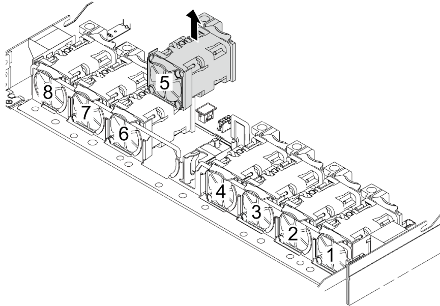
圖例 277. 卸下系統風扇
