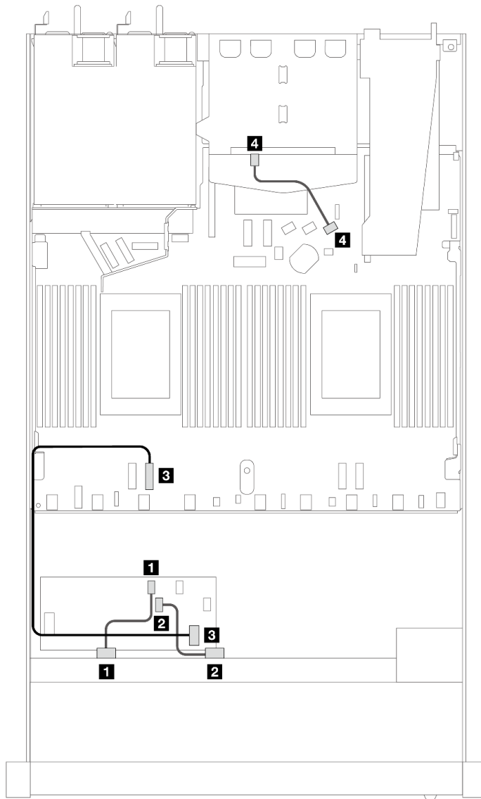
圖例 430. 配備 8i CFF RAID 配接卡 (Gen 3) (已安裝 2 x 2.5 SAS/SATA 硬碟) 之 8 x 2.5 吋前方 SAS/SATA 機槽的纜線佈線
