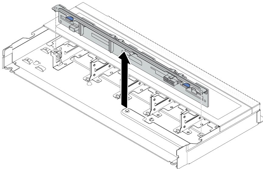
圖例 13. 卸下十個 2.5 吋熱抽換硬碟的背板
