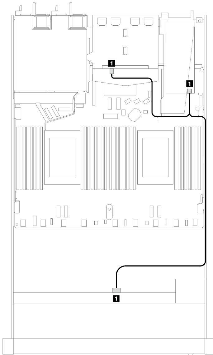
圖例 361. 配備 8i SFF RAID 配接卡 (Gen 4) 和後方 2 x 2.5 吋 SAS/SATA 硬碟之 4 x 3.5 吋前方 SAS/SATA 機槽的纜線佈線
