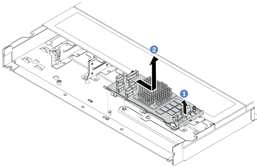
圖例 88. 卸下內部 CFF RAID 配接卡
