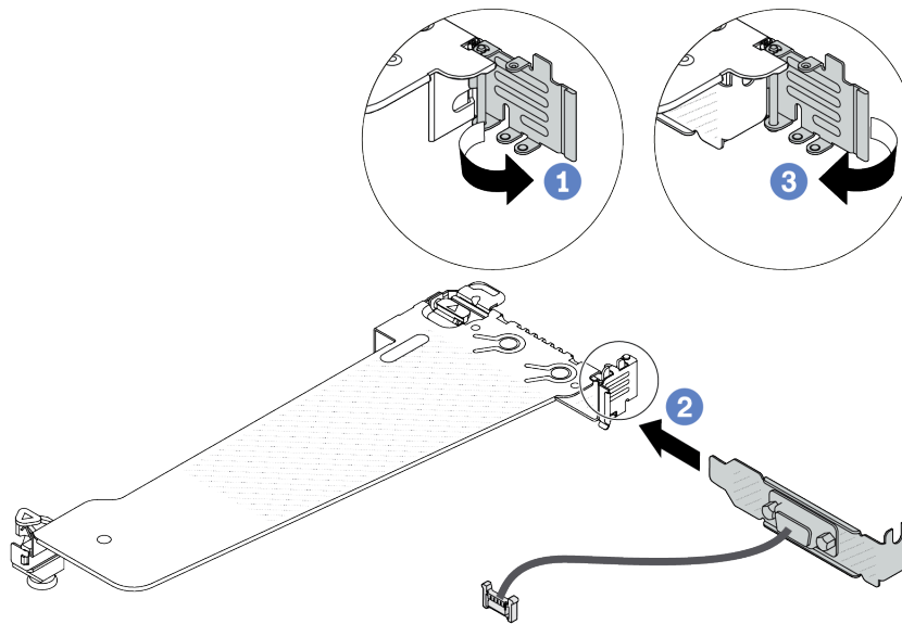
圖例 265. 安裝序列埠模組
