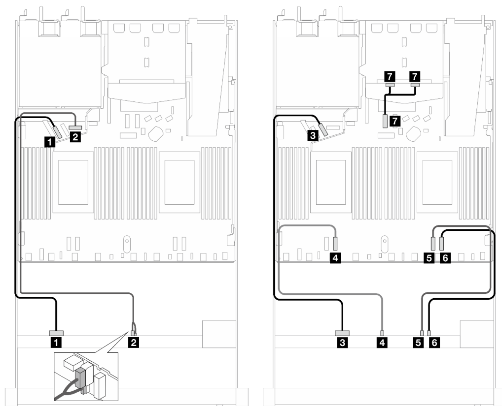
圖例 473. 12 x 2.5 吋 NVMe 前方硬碟機載配置的纜線佈線
