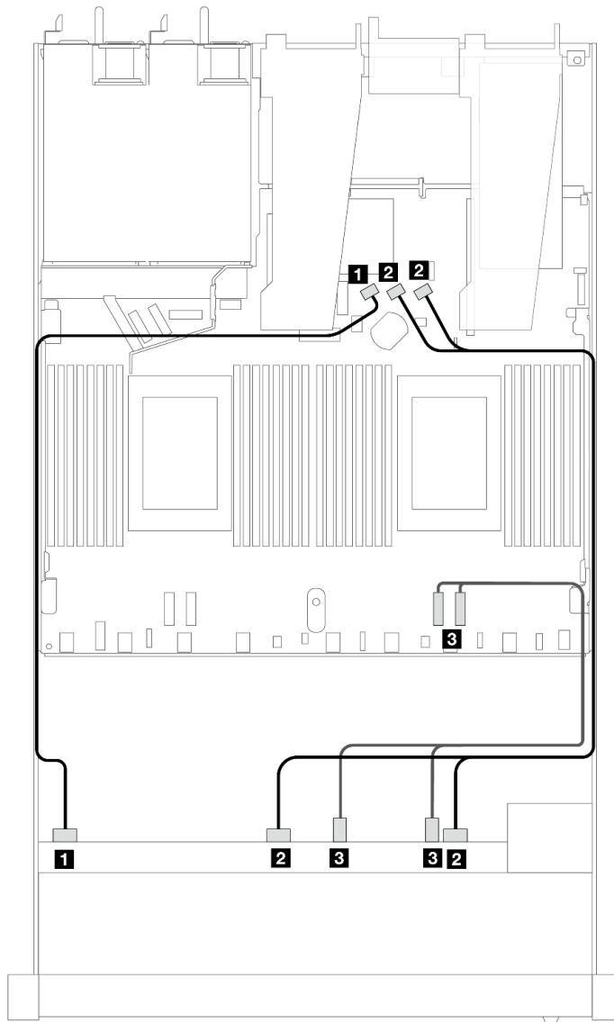
圖例 433. 6 個前方 SAS/SATA 硬碟和 4 個前方 AnyBay 機槽機載配置的纜線佈線
