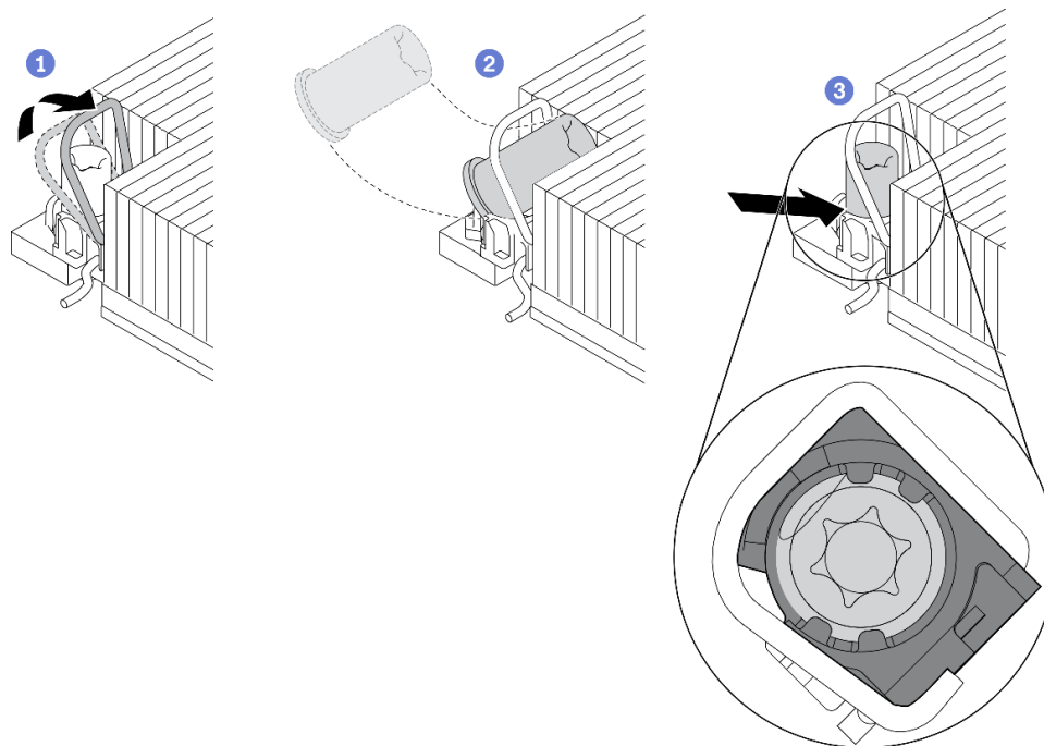
圖例 72. 將 Torx T30 螺帽安裝到散熱槽
