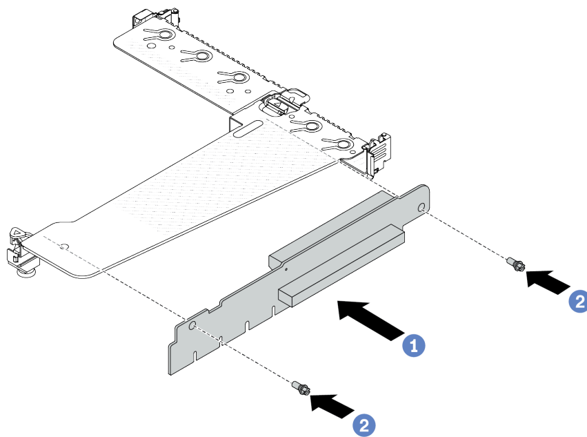
圖例 254. 擴充卡安裝
