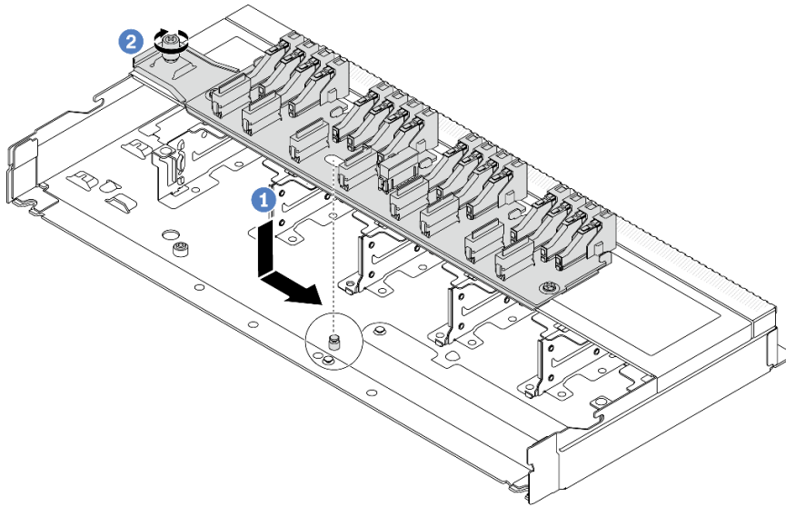
圖例 18. 安裝 16-EDSFF 硬碟背板
