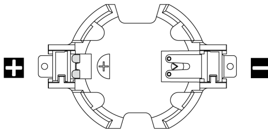
圖例 27. CMOS 電池插座上的正極和負極
