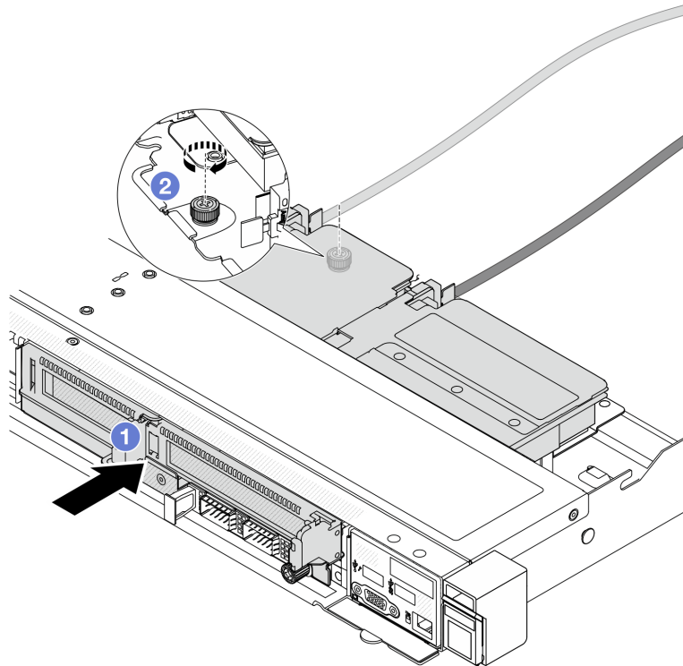
圖例 39. 安裝正面擴充卡匣
