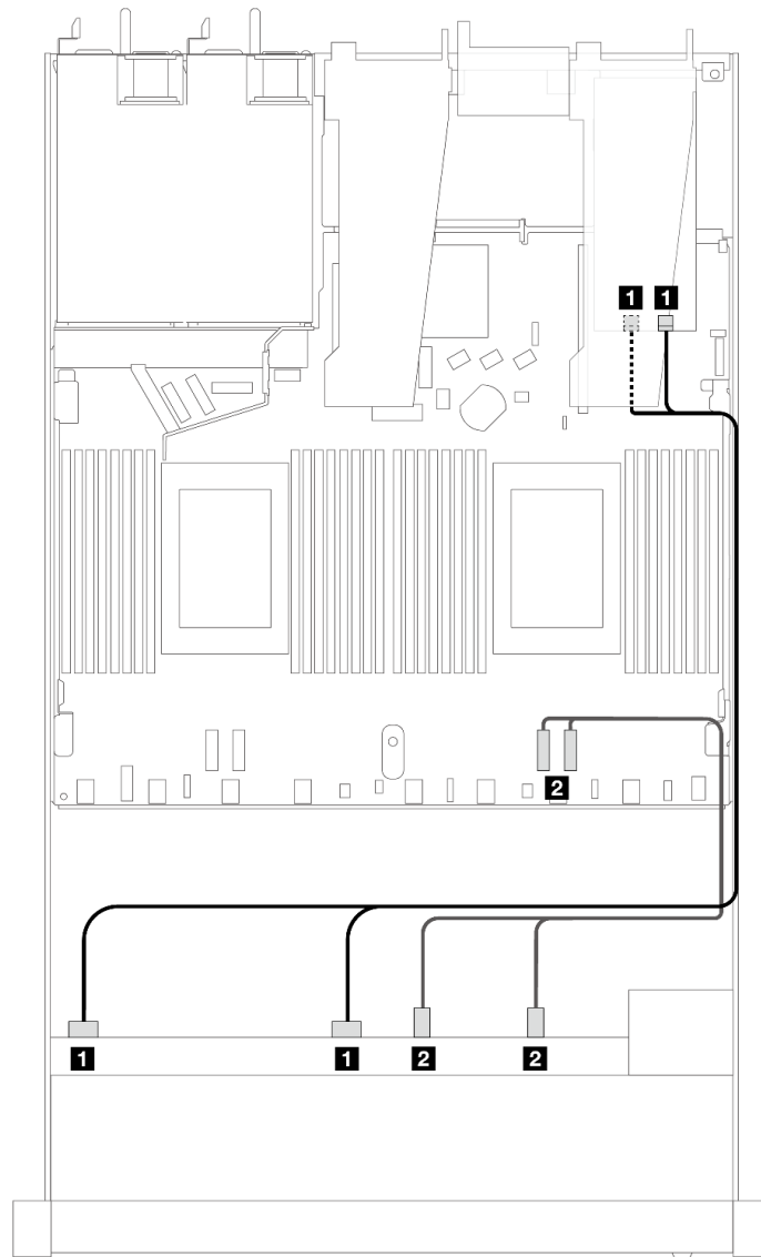
圖例 387. 包含 8i 或 16i SFF RAID 配接卡 (Gen 3) 的 6 個 SAS/SATA 硬碟和 2 個 AnyBay 硬碟和 2 個 NVMe 前方機槽的纜線佈線
