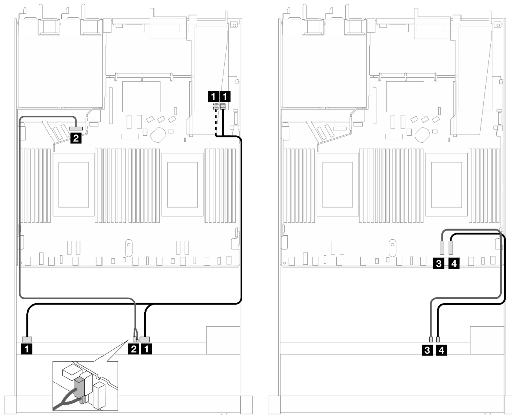
圖例 467. 包含 16i SFF RAID 配接卡 (Gen 3) 的六個 SAS/SATA 硬碟和兩個 AnyBay 硬碟和兩個 NVMe 前方機槽的纜線佈線
