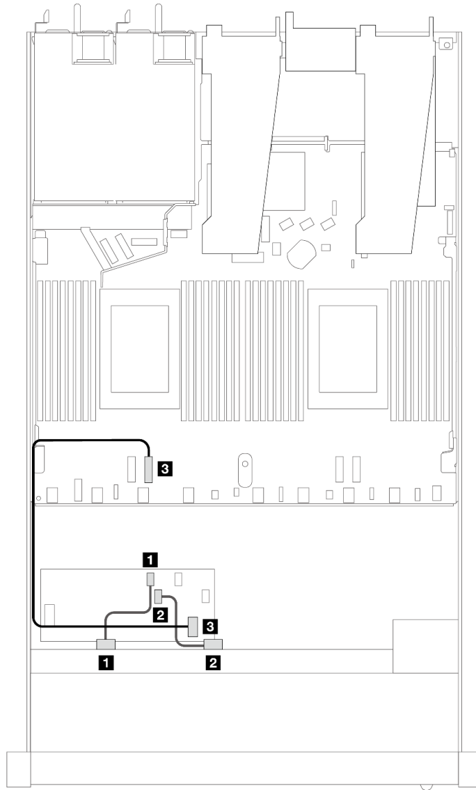
圖例 429. 包含 8i 或 16i CFF RAID 配接卡 ( Gen 3 或 Gen 4 ) 的 8 x 2.5 吋前方 SAS/SATA 機槽的纜線佈線
