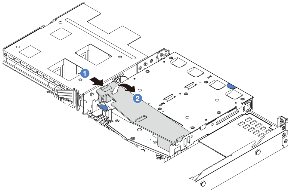
圖例 204. 卸下空氣擋板
