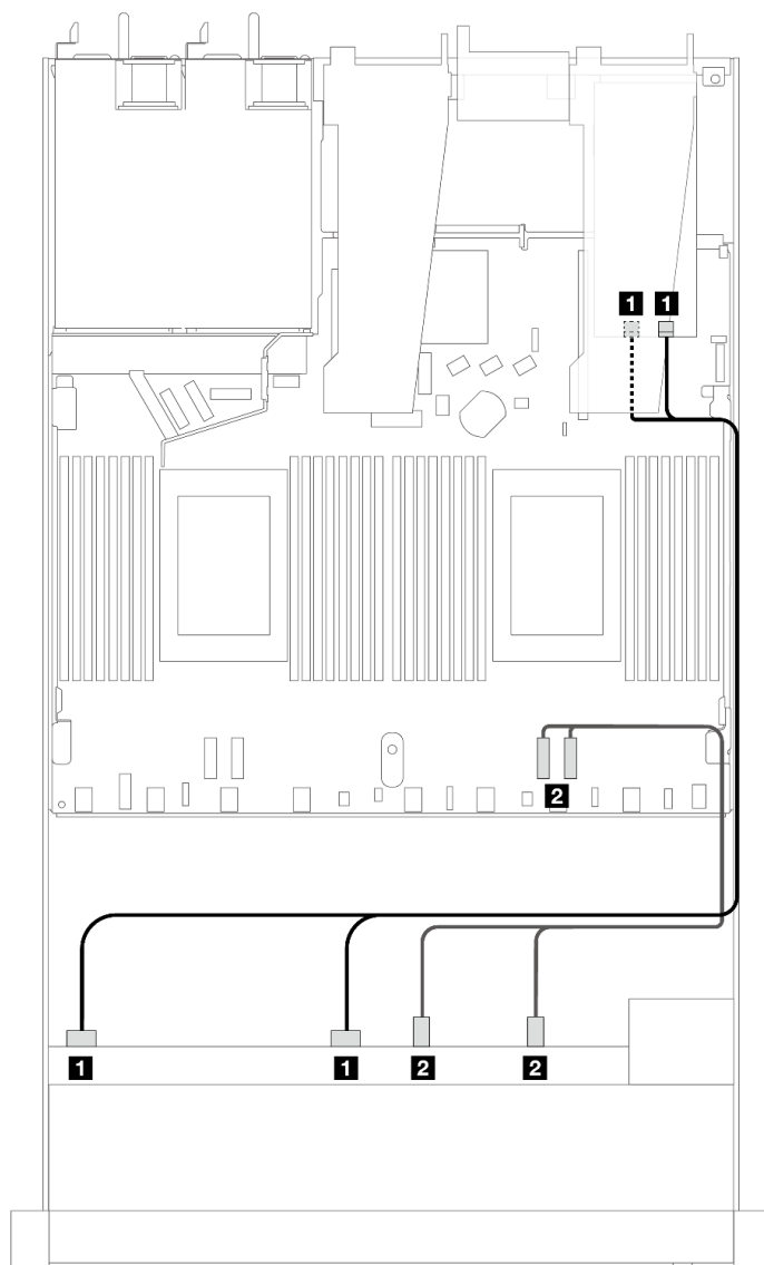
圖例 443. 包含 8i 或 16i SFF RAID 配接卡 (Gen 3) 的 6 個 SAS/SATA 硬碟和 2 個 AnyBay 硬碟和 2 個 NVMe 前方機槽的纜線佈線
