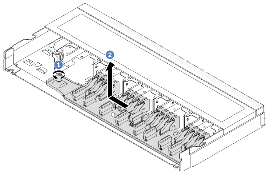
圖例 17. 卸下 16-EDSFF 硬碟背板
