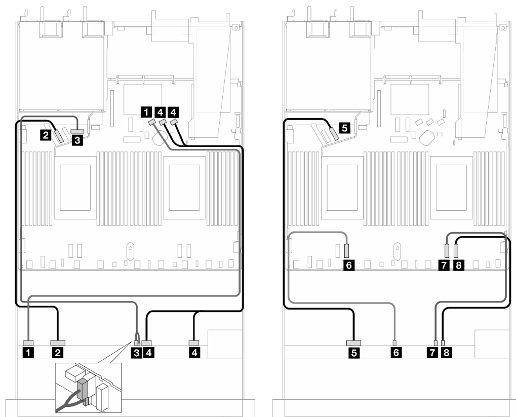
圖例 469. 10 x 2.5 吋 AnyBay 前方硬碟載配置的纜線佈線
