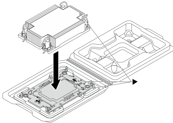
圖例 186. 將 PHM 和處理器裝到運送匣中
