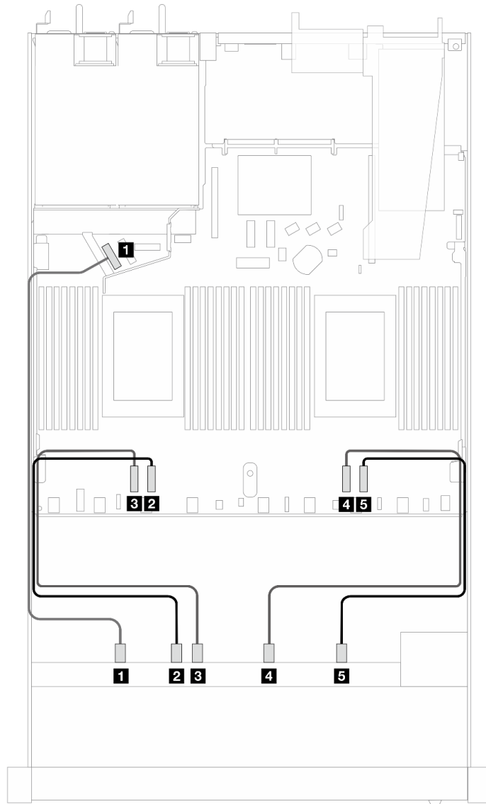
圖例 349. 用於液冷的 10 個 NVMe 磁碟機 ( Gen 4 背板 ) 的機載佈線
