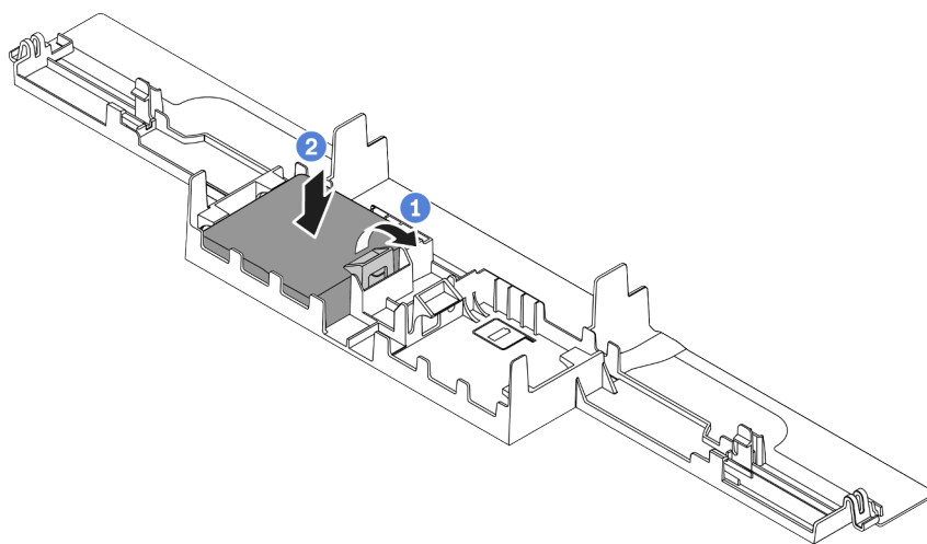
圖例 200. 將 RAID 快閃記憶體電源模組安裝在空氣擋板上
