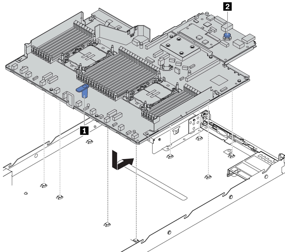
圖例 276. 安裝主機板組件
