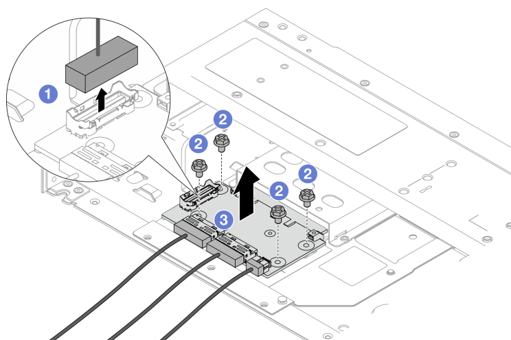
圖例 50. 卸下正面 OCP 轉插卡
