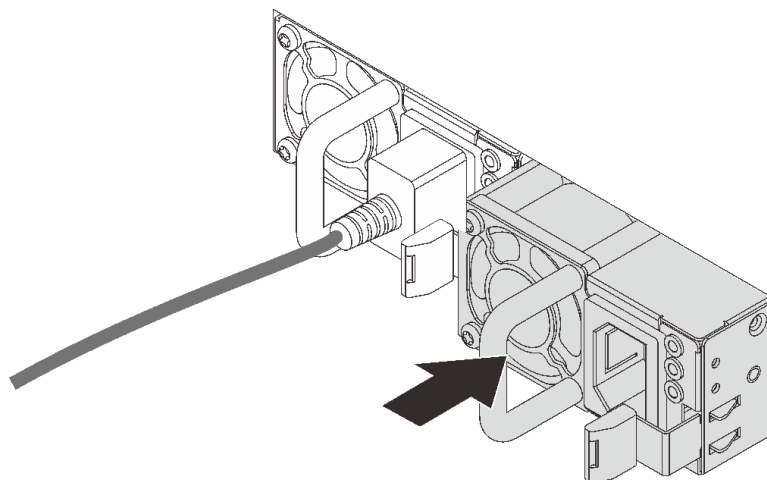
圖例 87. 安裝熱抽換電源供應器
