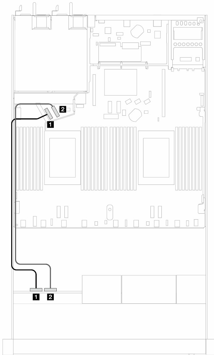
圖例 412. 4 x 2.5 吋前方 NVMe 磁碟機機載配置的纜線佈線
