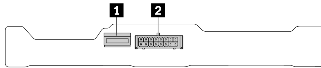
圖例 294. 後方 2 x 2.5 吋 NVMe 背板
