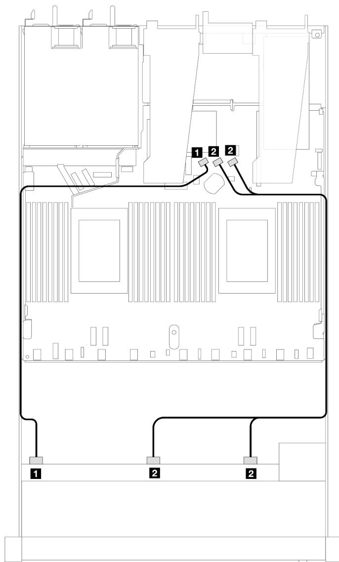
圖例 388. 10 x 2.5 SAS/SATA 前方硬碟機載配置的纜線佈線
