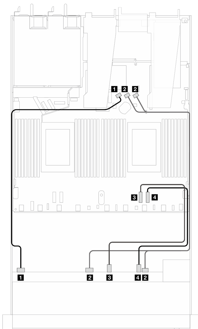
圖例 333. 六個 SAS/SATA 和四個 NVMe 前方硬碟機載配置的纜線佈線
