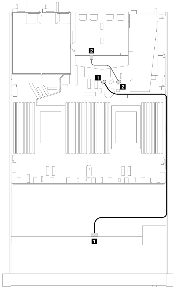
圖例 397. 配備 2 x 2.5 後方 SAS/SATA 硬碟之 4 x 3.5 吋前方 SAS/SATA 機槽機載配置的纜線佈線
