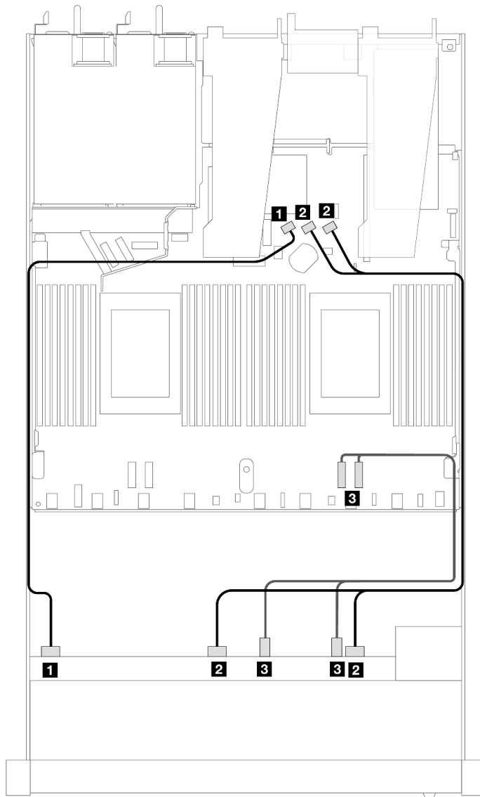
圖例 379. 6 個前方 SAS/SATA 硬碟和 4 個前方 AnyBay 機槽機載配置的纜線佈線
