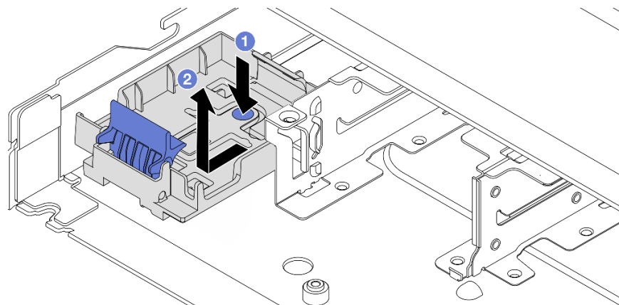
圖例 195. 卸下 RAID 快閃記憶體電源模組匣
