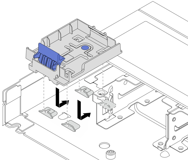
圖例 197. 安裝 RAID 快閃記憶體電源模組匣
