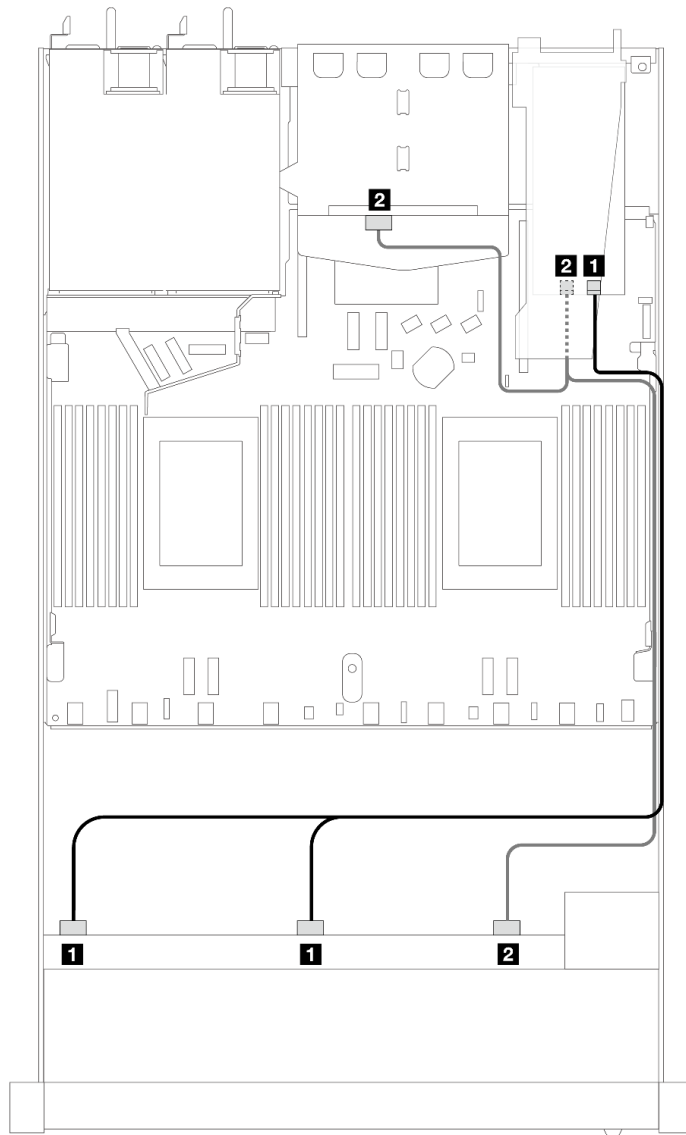
圖例 390. 安裝 2 x 2.5 後方 SAS/SATA 硬碟之 10 個前方 SAS/SATA 機槽和 16i SFF RAID 配接卡 (Gen 4) 的纜線佈線
