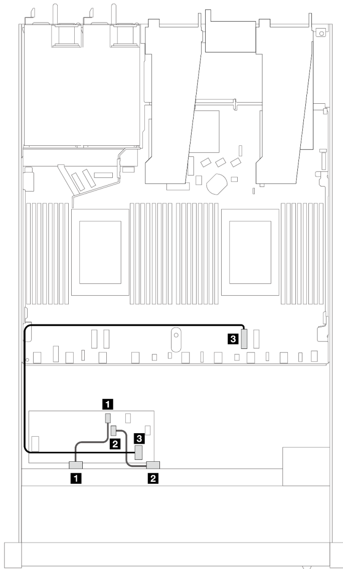
圖例 374. 包含 8i 或 16i CFF RAID 配接卡 (Gen 3) 的 8 x 2.5 吋前方 SAS/SATA 機槽的纜線佈線
