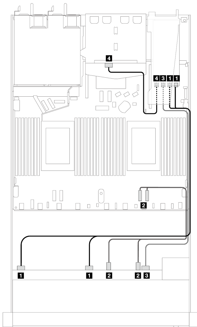
圖例 384. 6 個前方 SAS/SATA 硬碟和 4 個前方 AnyBay 機槽以及 16i SFF RAID 配接卡 (Gen 3) ( 已安裝 2 x 2.5 後方 SAS/SATA 硬碟 ) 的纜線佈線
