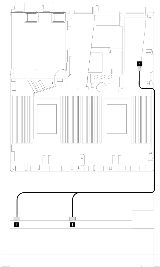
圖例 432. 包含 8i SFF RAID 配接卡 (Gen 4) 的 8 x 2.5 吋前方 U.3 硬碟纜線佈線
