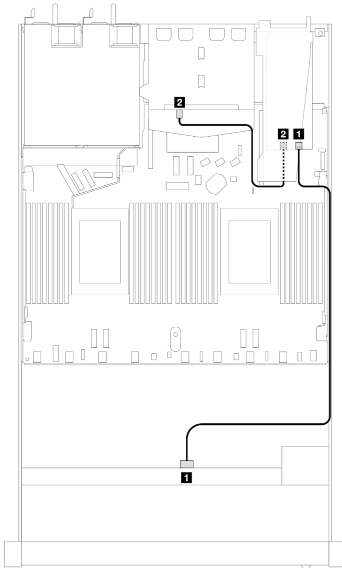
圖例 400. 配備 8i SFF RAID 配接卡 (Gen 3) 和後方 2 x 2.5 吋 SAS/SATA 硬碟之 4 x 3.5 吋前方 SAS/SATA 機槽的纜線佈線
