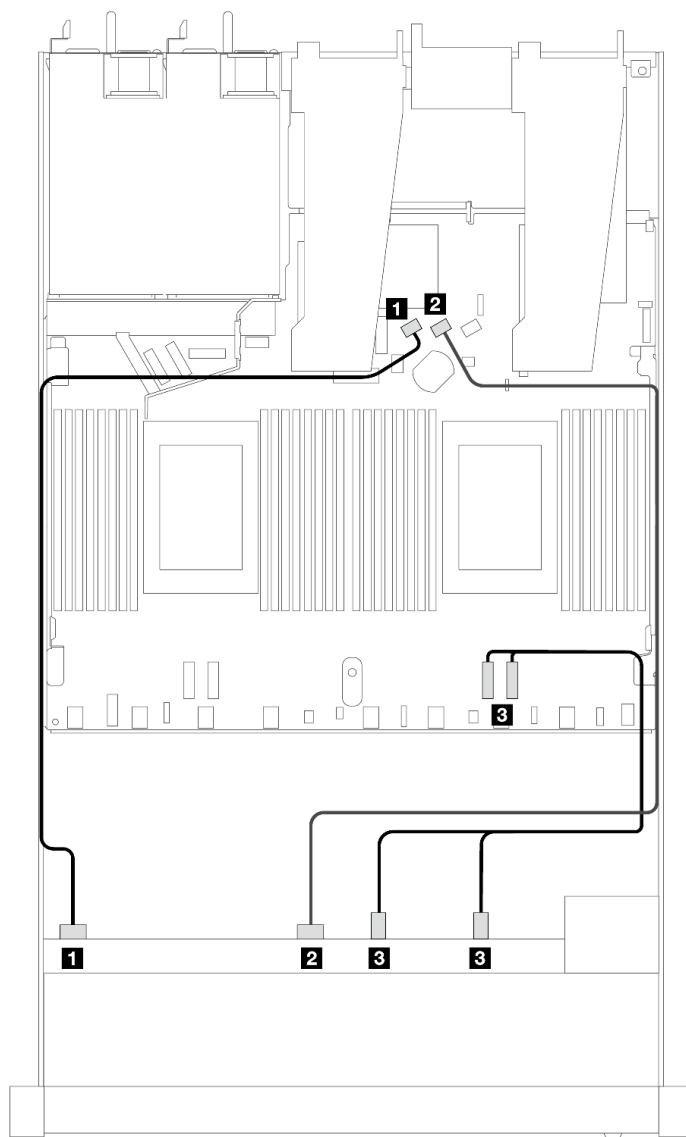
圖例 385. 6 個 SAS/SATA 硬碟和 2 個 AnyBay 和 2 個 NVMe 前方機槽機載配置的纜線佈線
