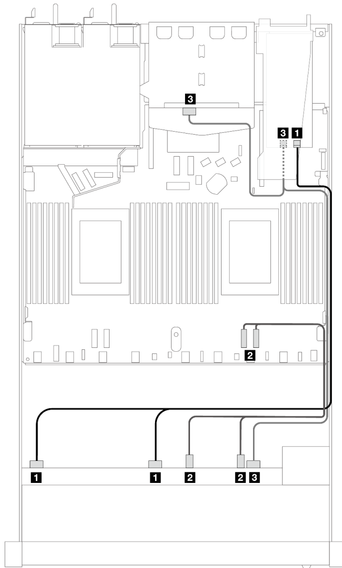
圖例 382. 6 個前方 SAS/SATA 硬碟和 4 個前方 AnyBay 機槽以及 16i SFF RAID 配接卡 (Gen 4) (已安裝 2 x 2.5 後方 SAS/SATA 硬碟) 的纜線佈線
