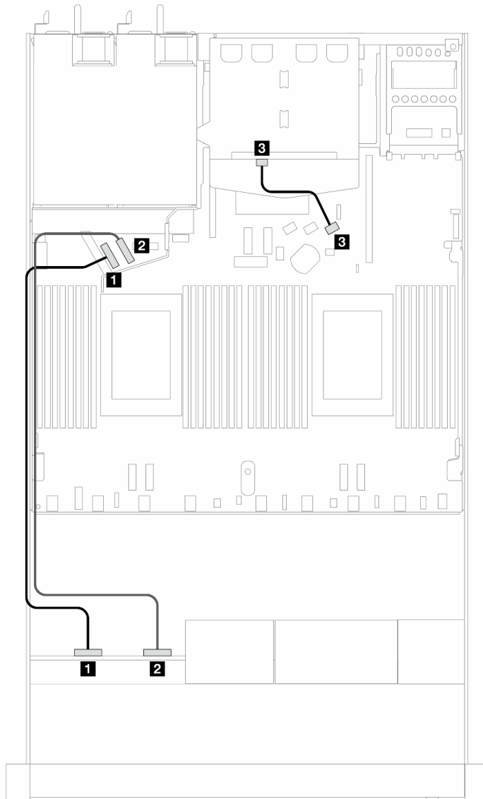
圖例 415. 4 x 2.5 吋前方 NVMe 磁碟機和 2 x 2.5 吋後方 SAS/SATA 硬碟機載配置的纜線佈線
