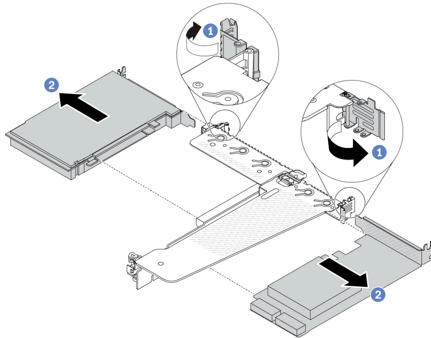
圖例 174. 從 LP-FH 擴充卡組件卸下 PCIe 配接卡
