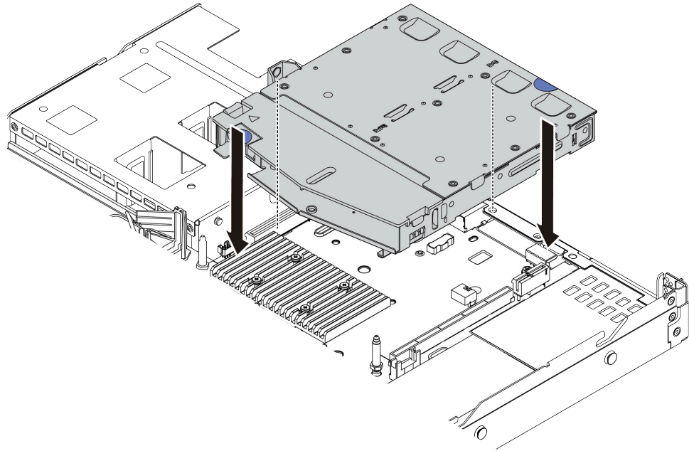
圖例 207. 安裝 2.5 吋背面框架
