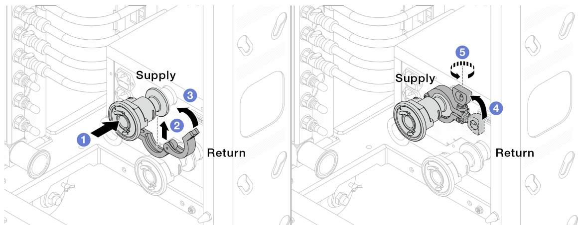
圖例 123. 安裝球閥
