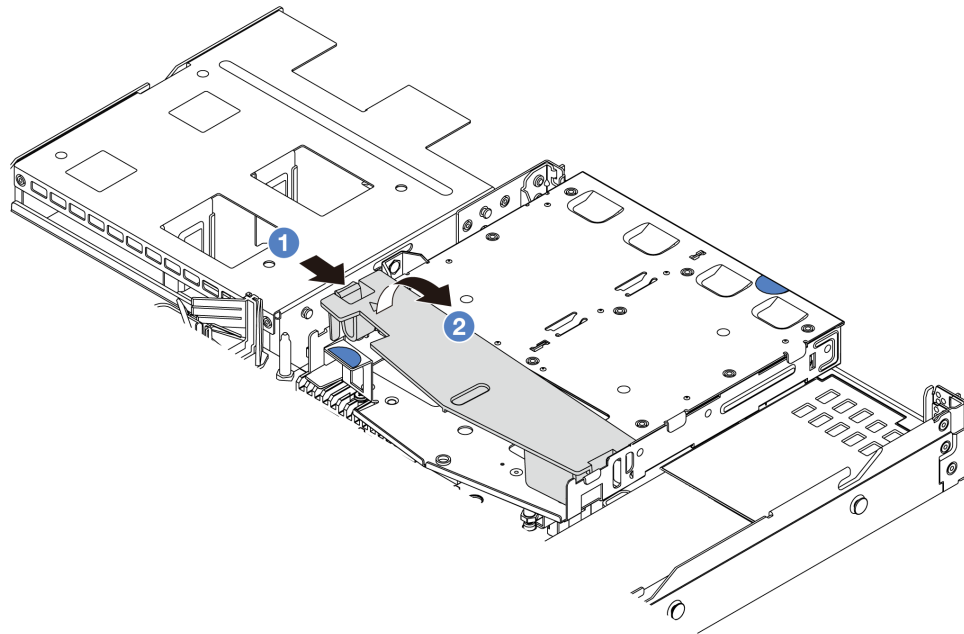
圖例 19. 卸下空氣擋板
