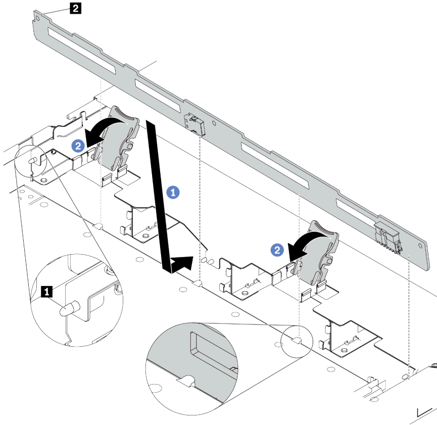
圖例 16. 安裝四個 3.5 吋熱抽換硬碟的背板
