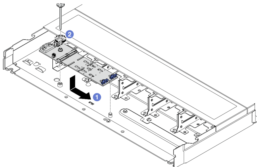
圖例 165. M.2 背板安裝
