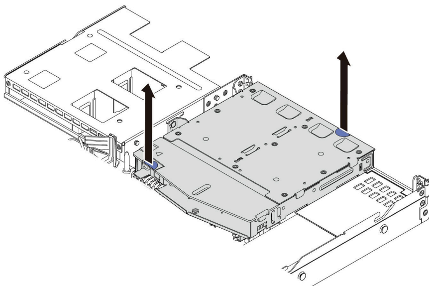
圖例 203. 卸下 2.5 吋背面框架
