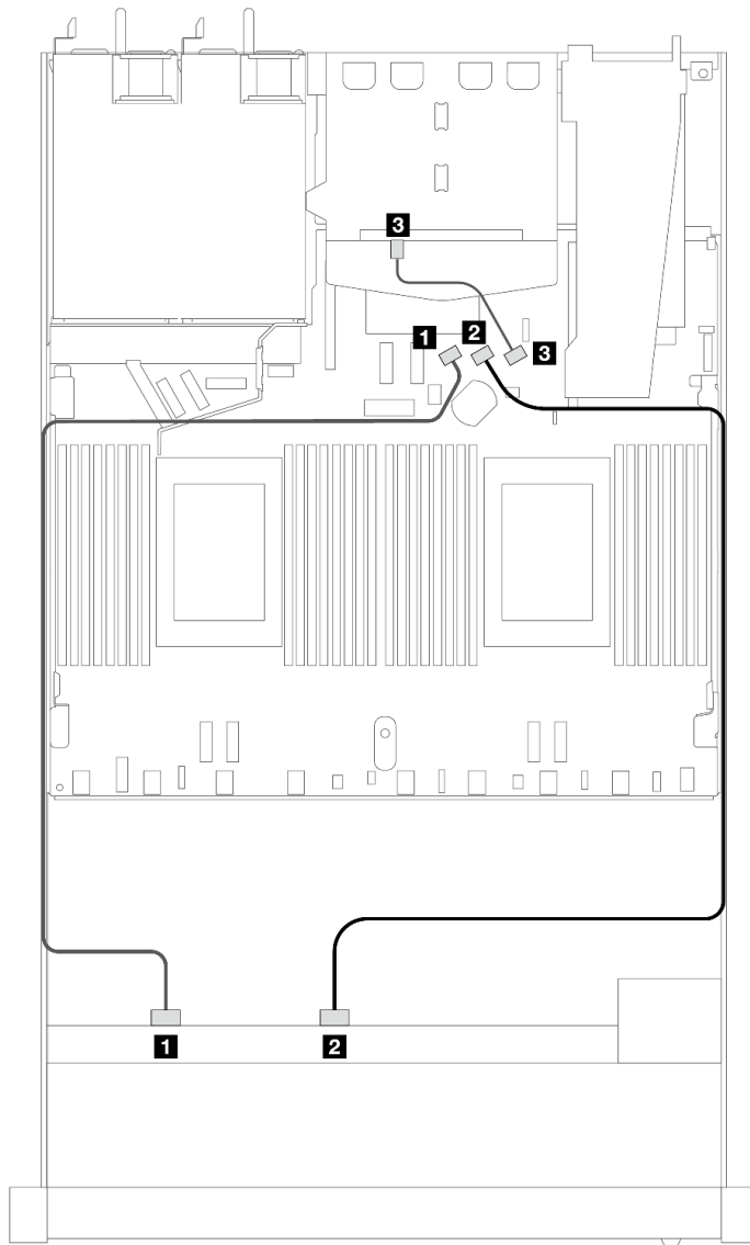
圖例 424. 安裝 2 x 2.5 後方 SAS/SATA 硬碟之 8 x 2.5 SAS/SATA 前方硬碟機載配置的纜線佈線
