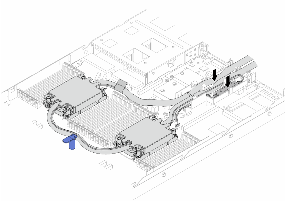
圖例 102. 放置水管和模組
