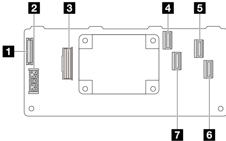
圖例 299. Gen 3 16i CFF RAID 配接卡 ( 四個埠接頭 )
