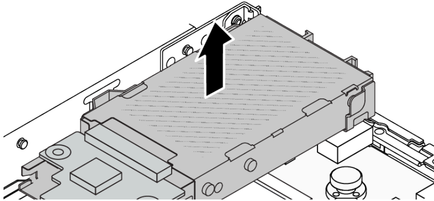
圖例 208. 卸下 7 公釐背面框架
