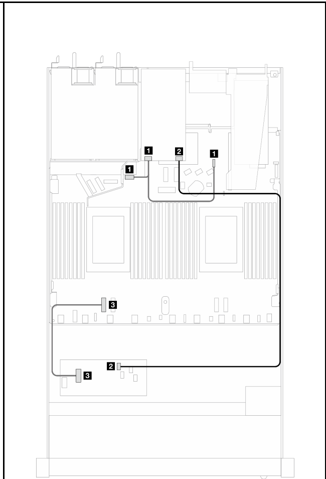
圖例 324. 7 公釐背板到 Gen 3/4 CFF RAID 配接卡
