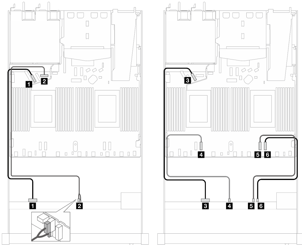
圖例 472. 10 x 2.5 吋 NVMe 前方硬碟機載配置的纜線佈線
