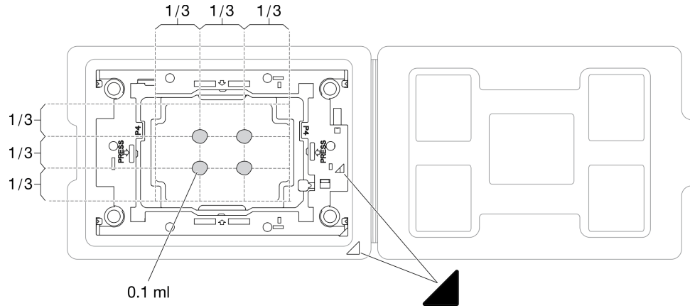
圖例 185. 運送匣中的處理器塗上散熱膏
