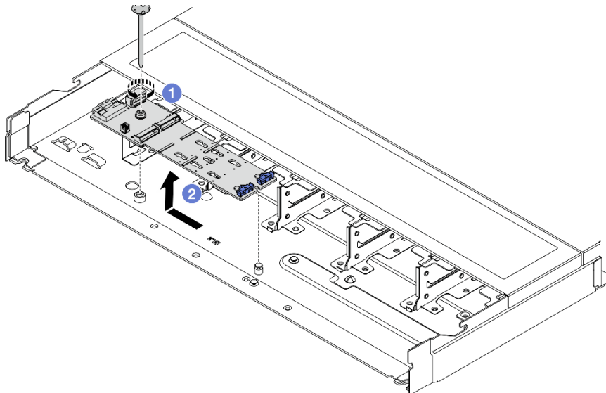
圖例 162. 卸下 M.2 模組
