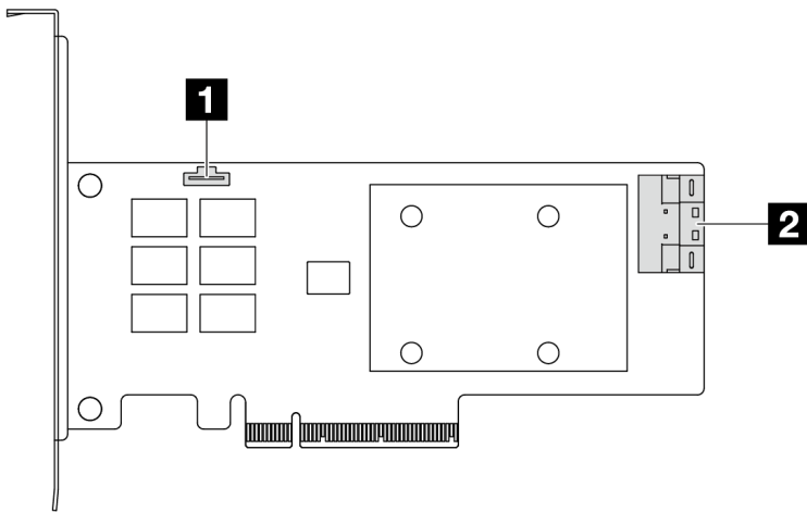
圖例 298. Gen 4 8i SFF RAID/HBA 配接卡 ( 一個埠接頭 )
