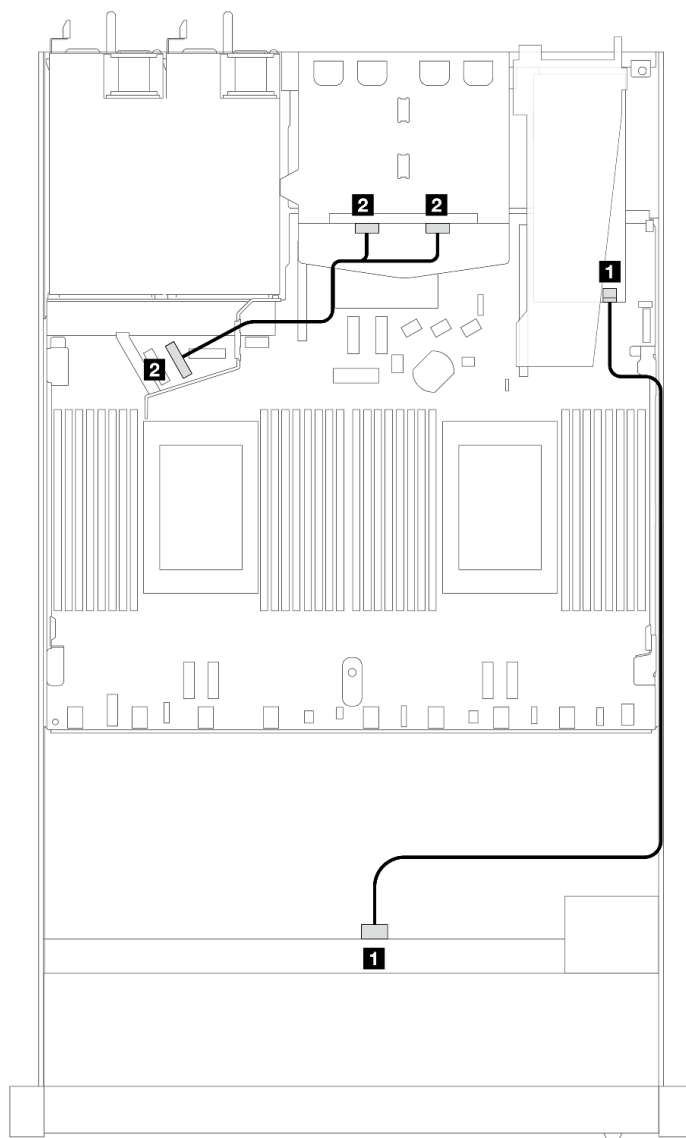
圖例 399. 配備 8i SFF RAID 配接卡和後方 2 x 2.5 吋 NVMe 硬碟之 4 x 3.5 吋前方 SAS/SATA 機槽的纜線佈線
