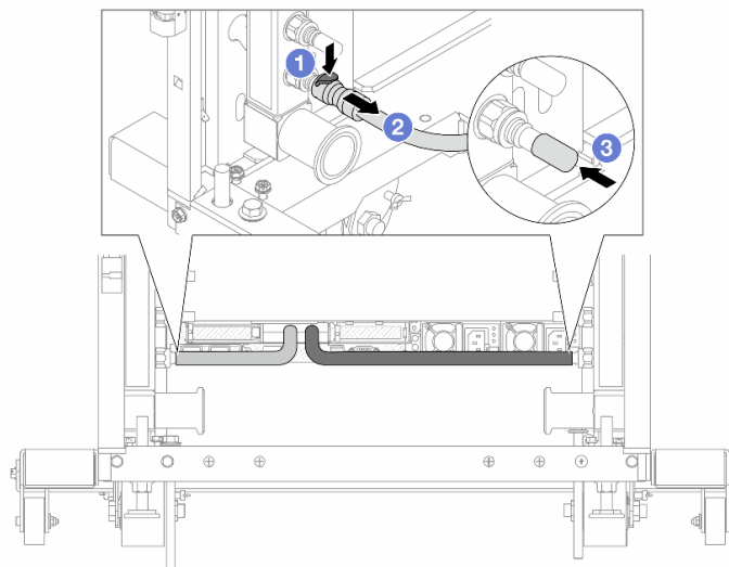
圖例 136. 移除 quick connect 插頭
