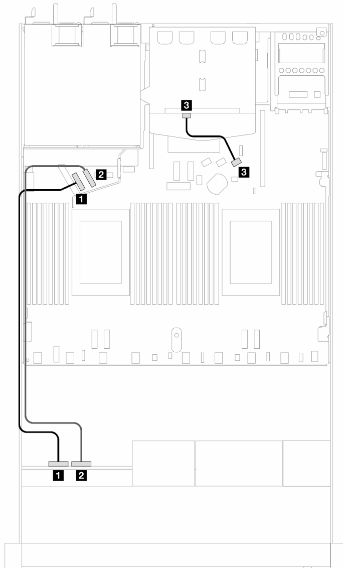
圖例 413. 4 x 2.5 吋前方 NVMe 磁碟機和 2 x 2.5 吋後方 SAS/SATA 硬碟機載配置的纜線佈線
