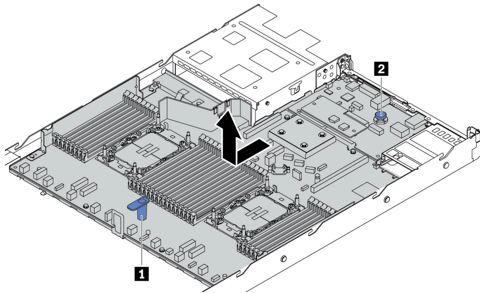
圖例 273. 卸下主機板組件
