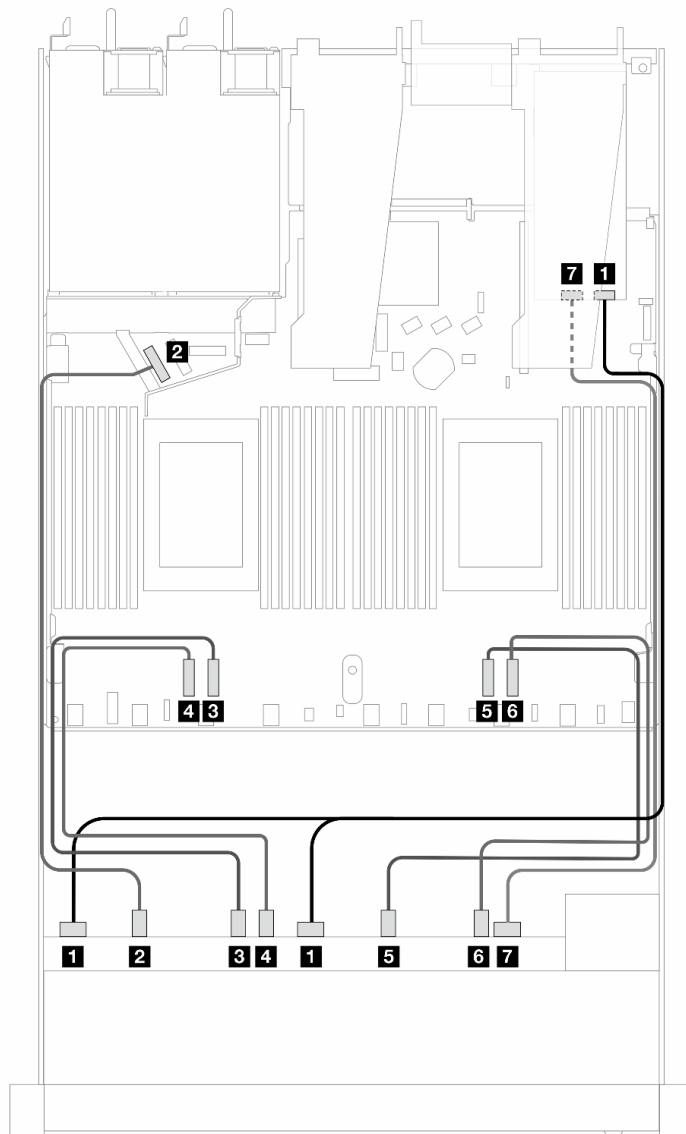
圖例 355. 包含 16i SFF RAID 配接卡 (Gen 4) 的 10 個前方 AnyBay 硬碟的纜線佈線
