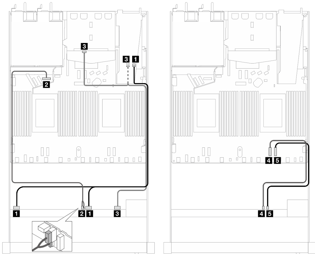
圖例 460. 六個前方 SAS/SATA 硬碟和四個前方 AnyBay 機槽以及 16i SFF RAID 配接卡 (Gen 4) (已安裝兩個後方 SAS/SATA 硬碟) 的纜線佈線
