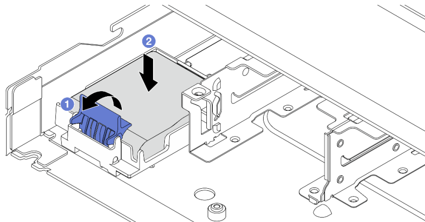
圖例 198. 將 RAID 快閃記憶體電源模組安裝在機箱
