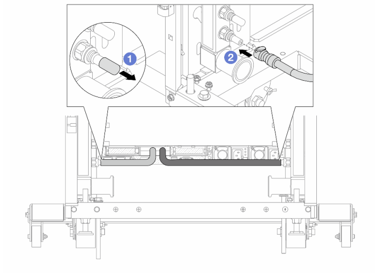
圖例 144. 安裝快速連接插件
