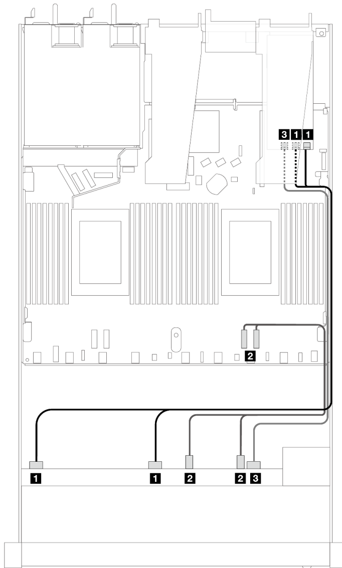
圖例 437. 包含 16i SFF RAID 配接卡 (Gen 3) 的 6 個前方 SAS/SATA 硬碟和 4 個前方 AnyBay 機槽的纜線佈線
