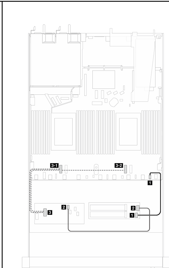
圖例 321. M.2 背板到 Gen 3/4 CFF RAID 配接卡
