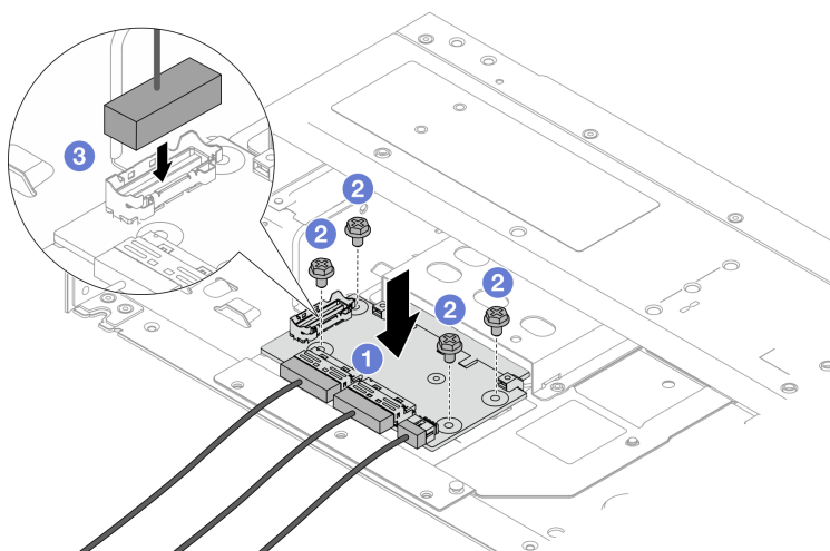
圖例 51. 安裝正面 OCP 轉插卡
