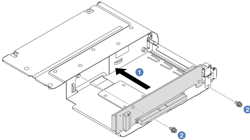
圖例 45. 將擴充卡安裝到全高匣
