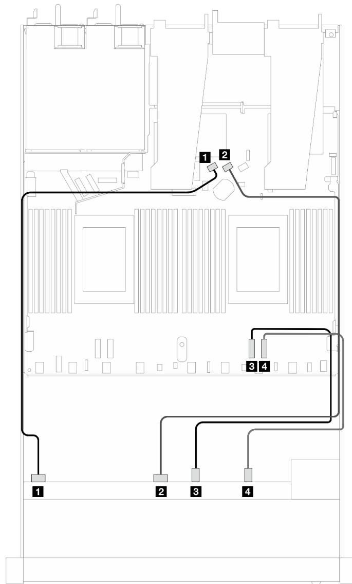
圖例 338. 六個 SAS/SATA 硬碟和兩個 AnyBay 和 兩個 NVMe 前方機槽機載配置的纜線佈線
