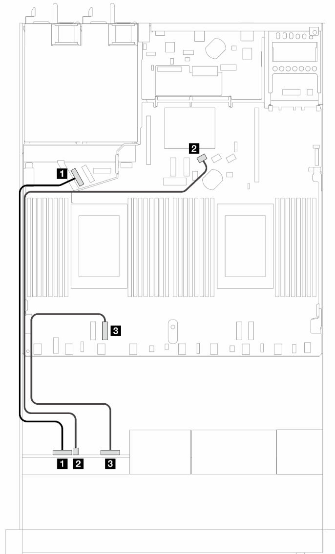
圖例 416. 4 x 2.5 吋前方 AnyBay 硬碟機載配置的纜線佈線
