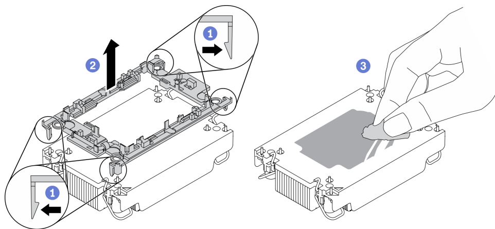
圖例 182. 將處理器支架與散熱槽分開
