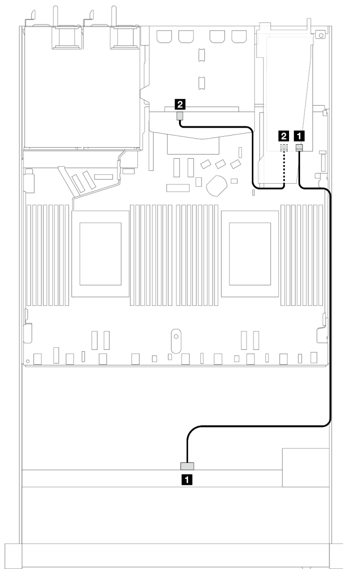
圖例 360. 配備 8i SFF RAID 配接卡 (Gen 3) 和後方 2 x 2.5 吋 SAS/SATA 硬碟之 4 x 3.5 吋前方 SAS/SATA 機槽的纜線佈線
