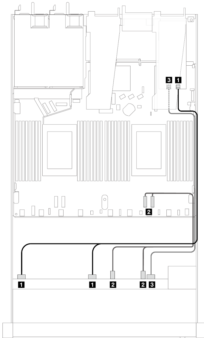
圖例 381. 包含 16i SFF RAID 配接卡 (Gen 4) 的 6 個前方 SAS/SATA 硬碟和 4 個前方 AnyBay 機槽的纜線佈線
