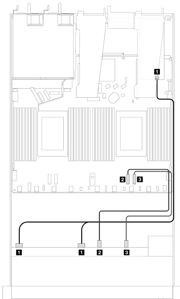
圖例 334. 包含 8i 或 16i SFF RAID 配接卡 (Gen 4) 的六個前方 SAS/SATA 硬碟和四個前方 AnyBay 機槽的纜線佈線
