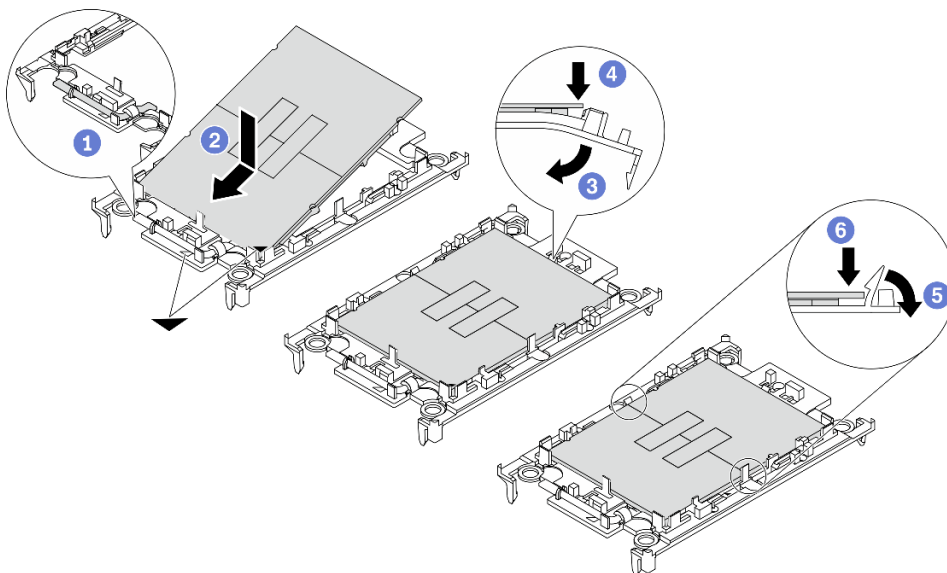
圖例 184. 安裝處理器支架
