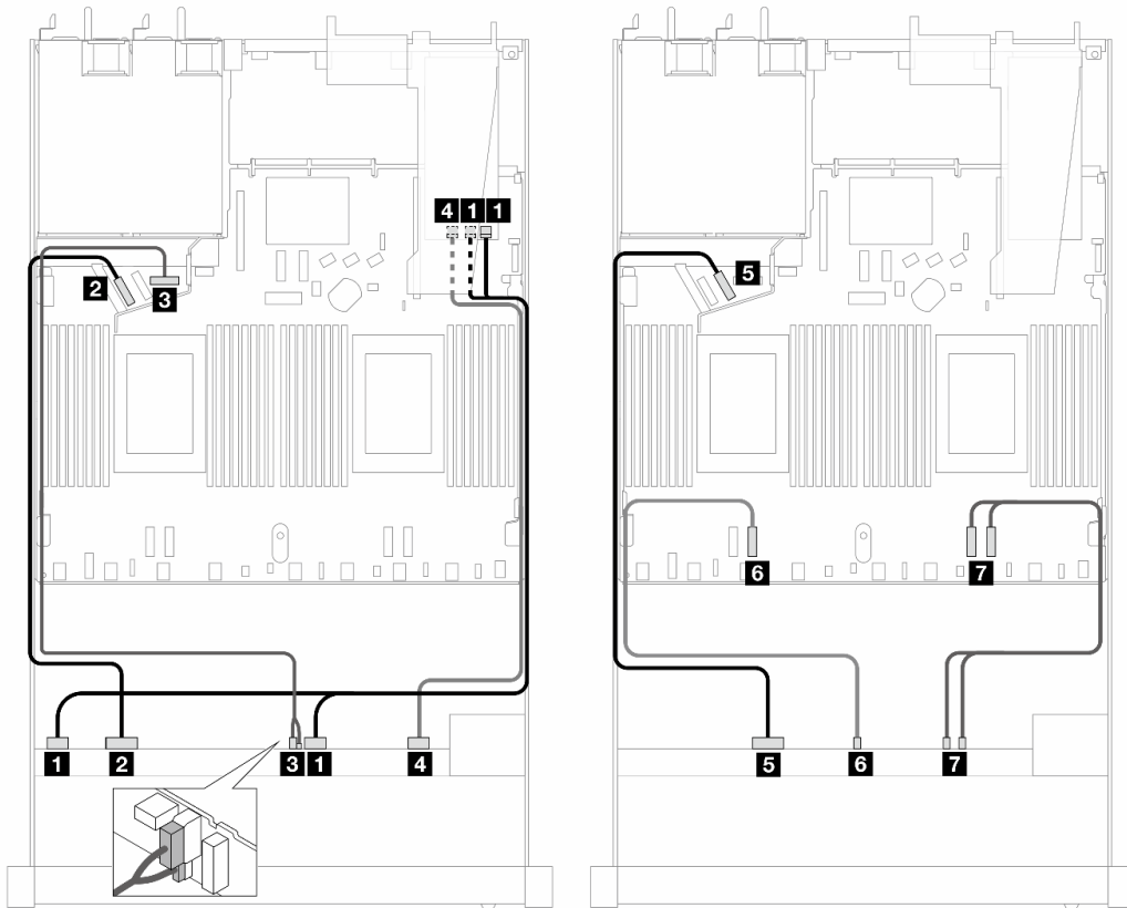
圖例 353. 包含 16i SFF RAID 配接卡 (Gen 3) 的 10 個 AnyBay 硬碟的纜線佈線
