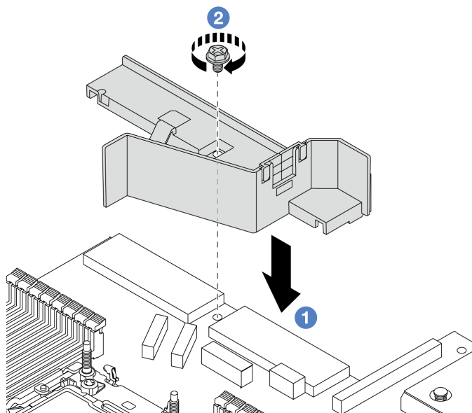
圖例 177. 安裝電源供應器空氣擋板
