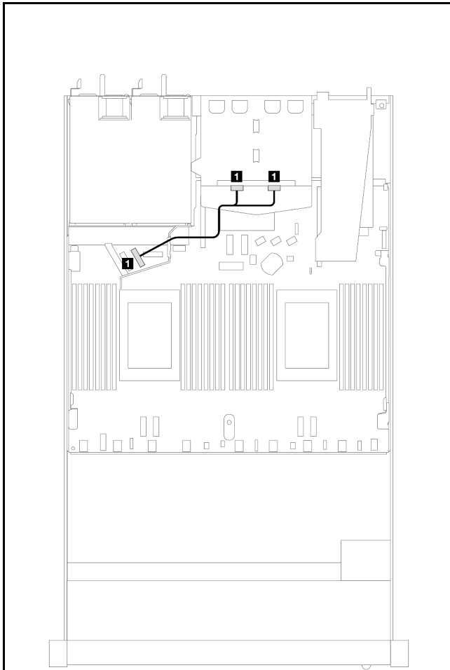
圖例 325. 安裝了兩個處理器的後方 NVMe 背板纜線佈線
