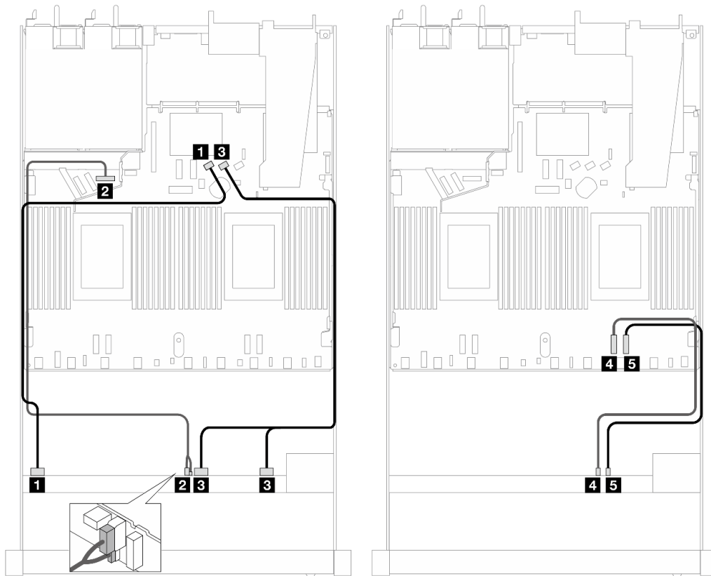
圖例 465. 六個 SAS/SATA 硬碟和兩個 AnyBay 和 兩個 NVMe 前方機槽機載配置的纜線佈線
