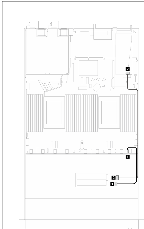
圖例 320. M.2 背板到 Gen 3/4 SFF RAID 配接卡
