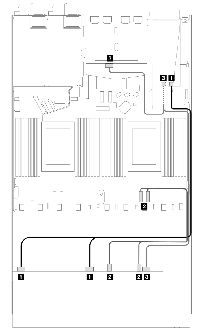
圖例 436. 6 個前方 SAS/SATA 硬碟和 4 個前方 AnyBay 機槽以及 16i SFF RAID 配接卡 (Gen 4) (已安裝 2 x 2.5 後方 SAS/SATA 硬碟) 的纜線佈線
