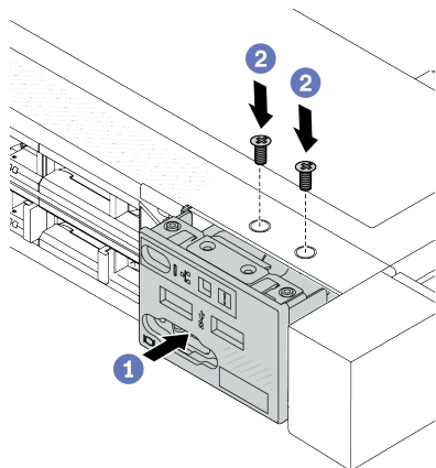
圖例 56. 將正面 I/O 模組安裝在 2.5 吋機箱上
