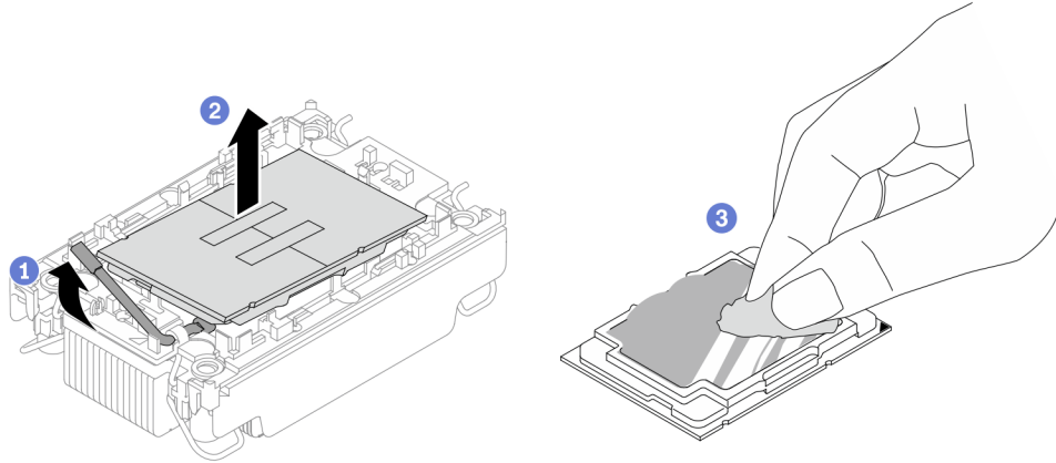
圖例 181. 將處理器與散熱槽和支架分開
