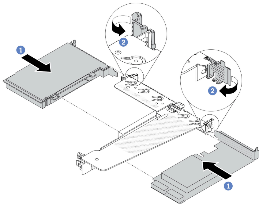
圖例 175. 將 PCIe 配接卡安裝在 LP-FH 擴充卡組件中
