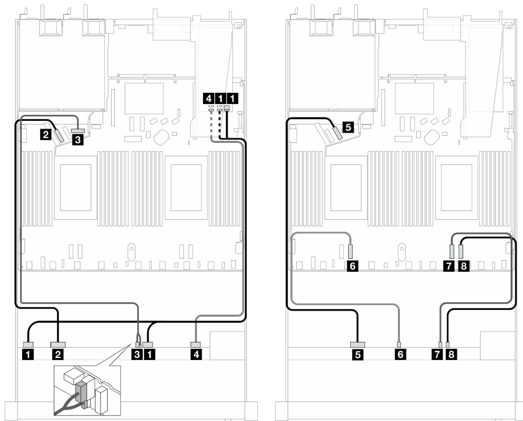
圖例 471. 包含 16i SFF RAID 配接卡 (Gen 3) 的 10 個 AnyBay 硬碟的纜線佈線
