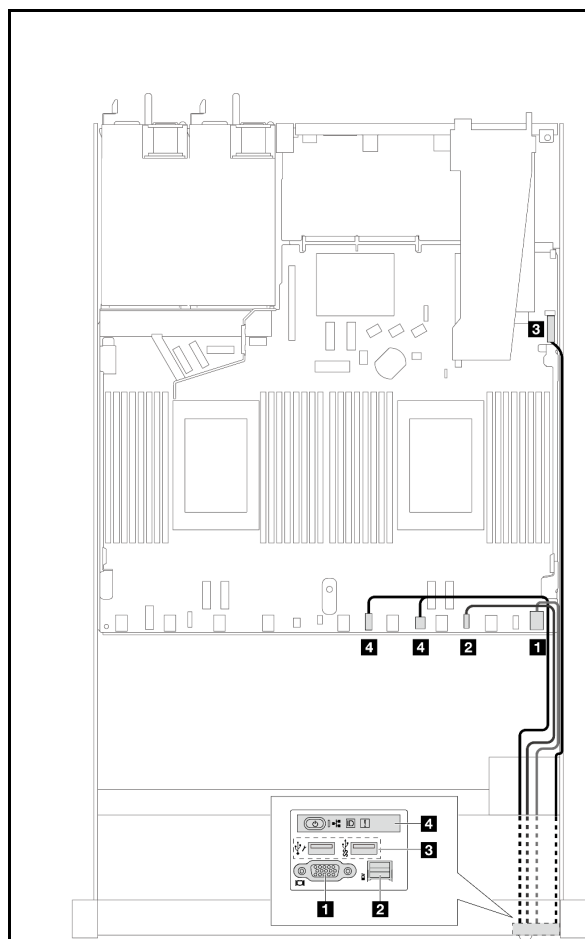
圖例 307. 2.5 吋機箱上正面 I/O 模組的纜線佈線
