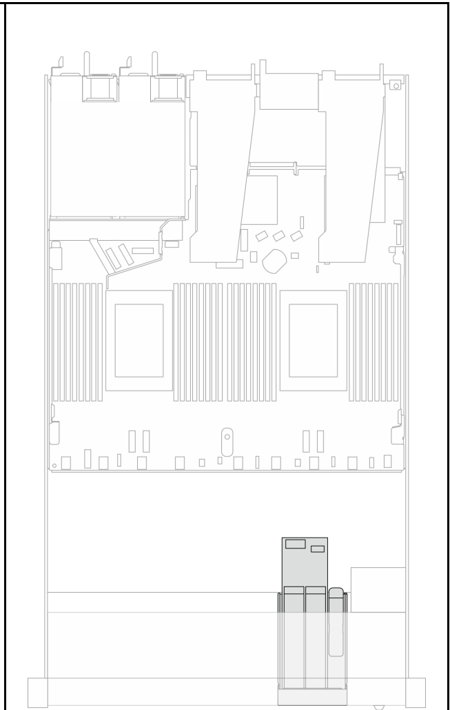
圖例 319. 16-EDSFF 硬碟機箱中的 M.2 硬碟組件
