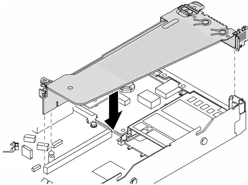
圖例 266. 安裝擴充卡組件
