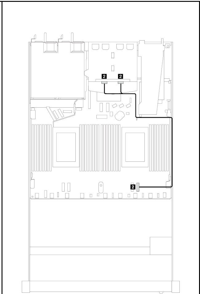
圖例 326. 安裝了一個處理器的後方 NVMe 背板纜線佈線
