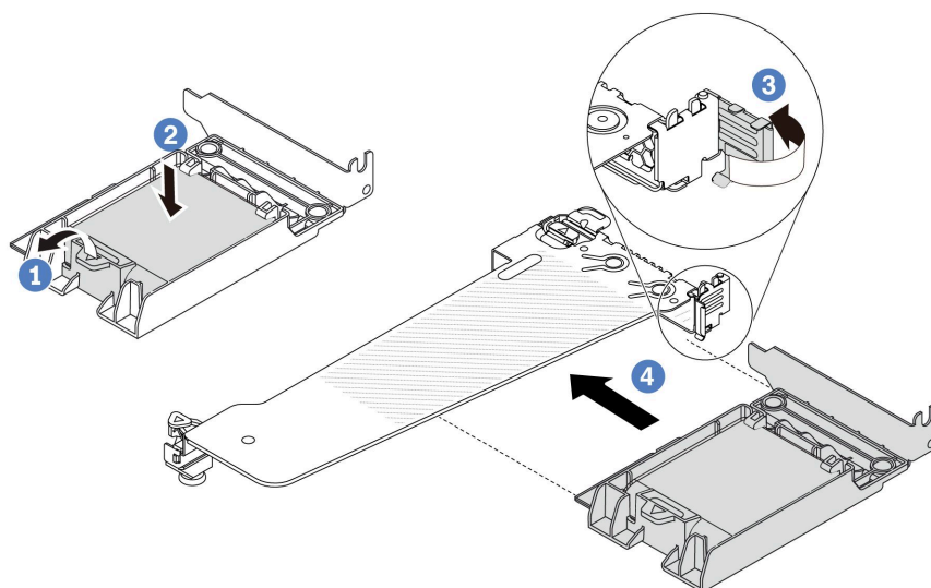
圖例 202. 將 RAID 快閃記憶體電源模組安裝在擴充卡上
