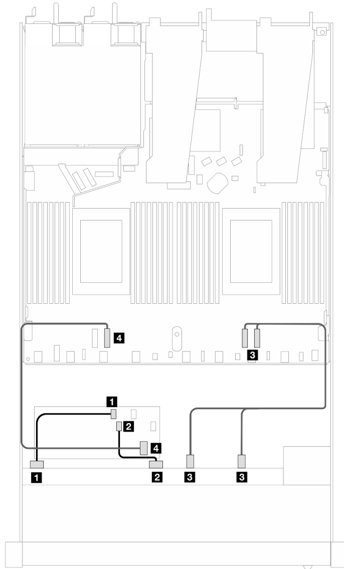
圖例 439. 包含 16i CFF RAID 配接卡 ( Gen 3 或 Gen 4 ) 的 6 個前方 SAS/SATA 硬碟和 4 個前方 AnyBay 機槽的纜線佈線
