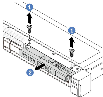
圖例 55. 卸下 3.5 吋機箱上的正面 I/O 模組
