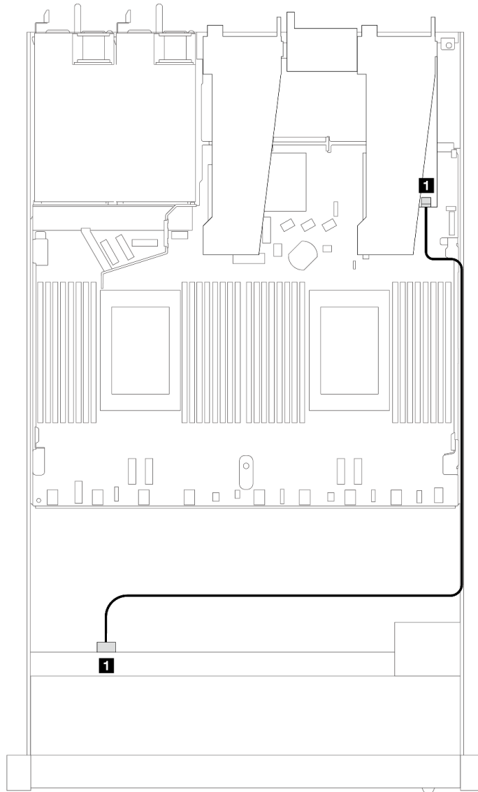
圖例 363. 包含 8i SFF RAID 配接卡的 4 x 2.5 吋前方 AnyBay 機槽的纜線佈線
