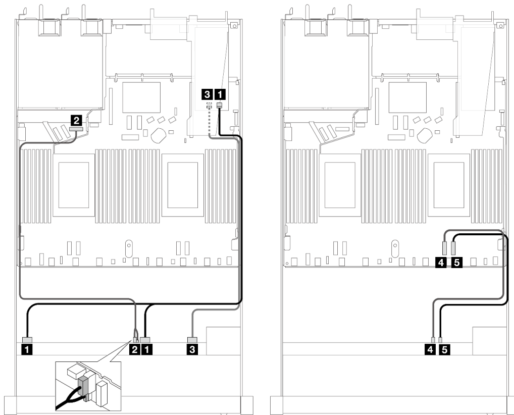
圖例 459. 包含 16i SFF RAID 配接卡 (Gen 4) 的六個前方 SAS/SATA 硬碟和四個前方 AnyBay 機槽的纜線佈線
