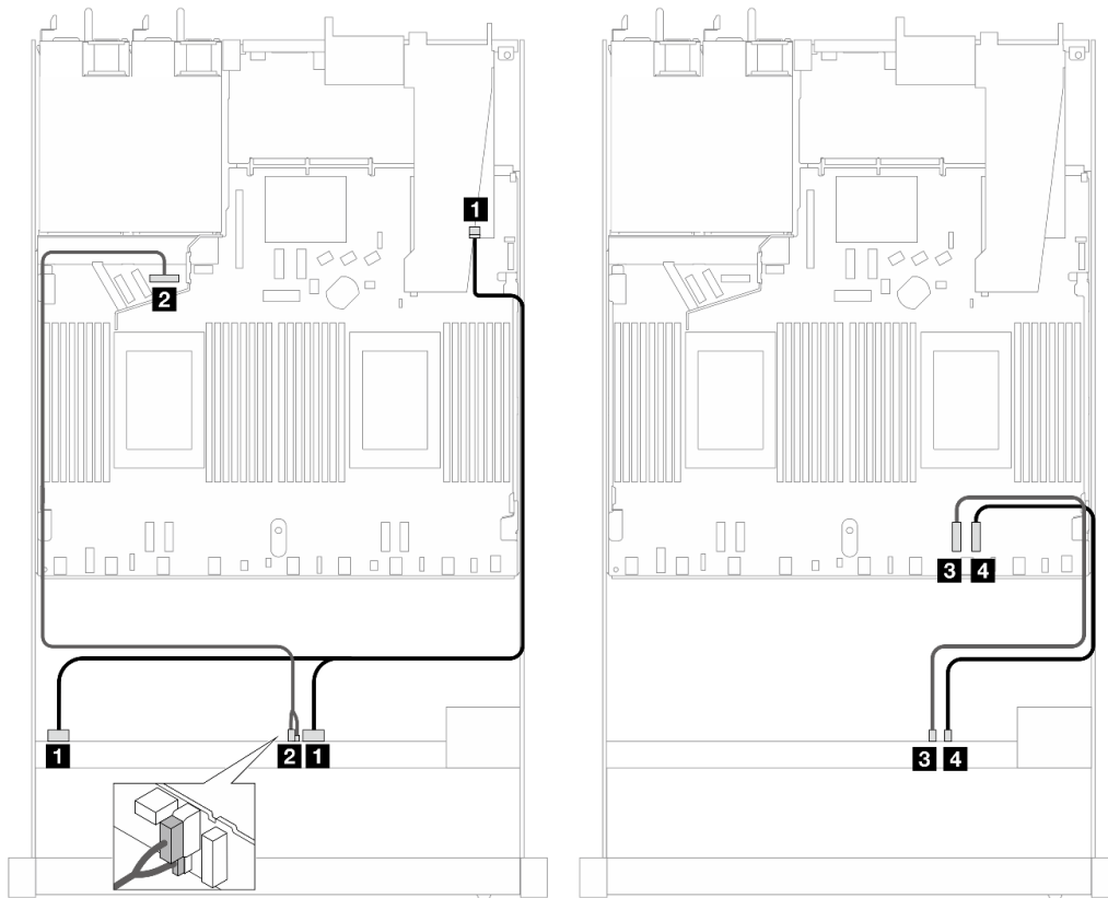
圖例 466. 包含 16i SFF RAID 配接卡 (Gen 4) 的六個 SAS/SATA 硬碟和兩個 AnyBay 硬碟和兩個 NVMe 前方機槽的纜線佈線
