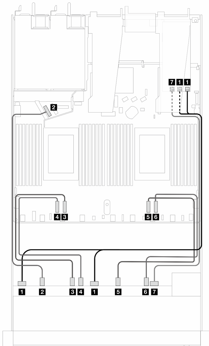
圖例 356. 包含 16i SFF RAID 配接卡 (Gen 3) 的 10 個 AnyBay 硬碟的纜線佈線
