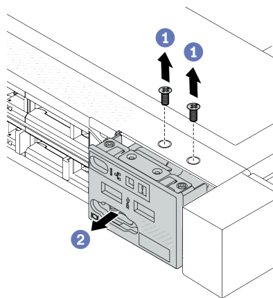
圖例 54. 卸下 2.5 吋機箱上的正面 I/O 模組
