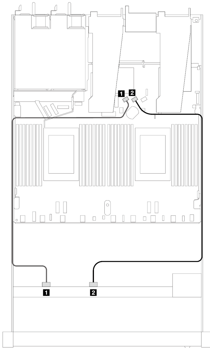
圖例 368. 8 x 2.5 SAS/SATA 前方硬碟機載配置的纜線佈線
