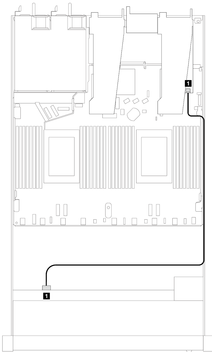
圖例 403. 包含 8i SFF RAID 配接卡的 4 x 2.5 吋前方 AnyBay 機槽的纜線佈線
