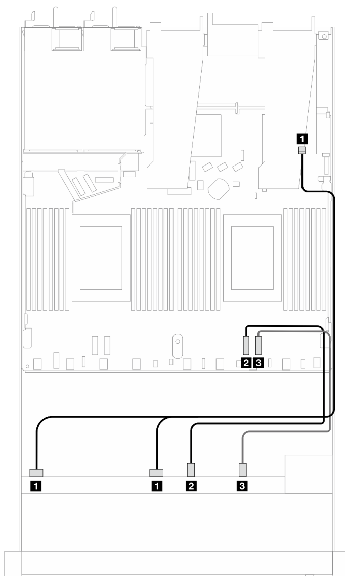
圖例 339. 包含 8i 或 16i SFF RAID 配接卡 (Gen 4) 的 6 個 SAS/SATA 硬碟和 2 個 AnyBay 硬碟和 2 個 NVMe 前方機槽的纜線佈線
