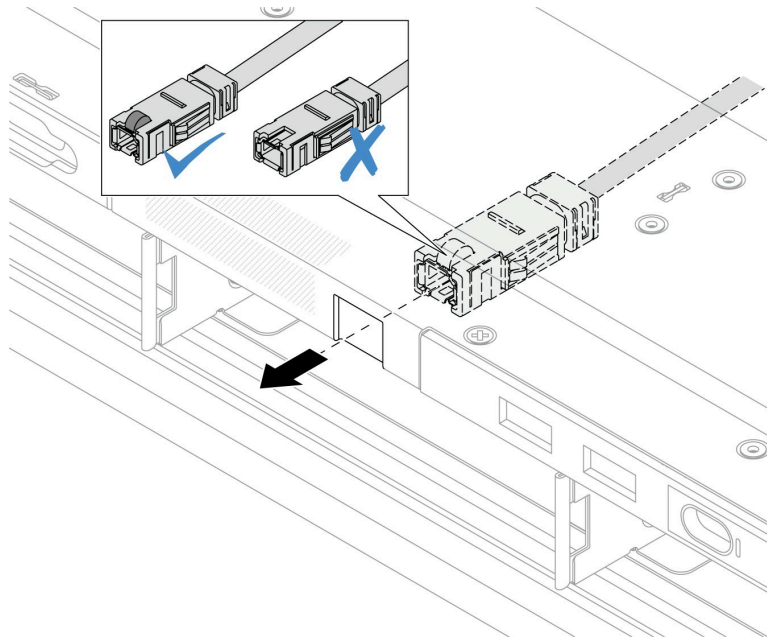
圖例 70. 外部 LCD 纜線的安裝
