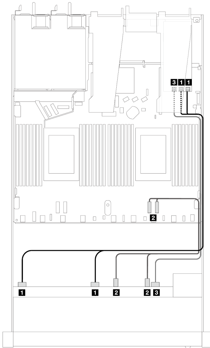
圖例 383. 包含 16i SFF RAID 配接卡 (Gen 3) 的 6 個前方 SAS/SATA 硬碟和 4 個前方 AnyBay 機槽的纜線佈線
