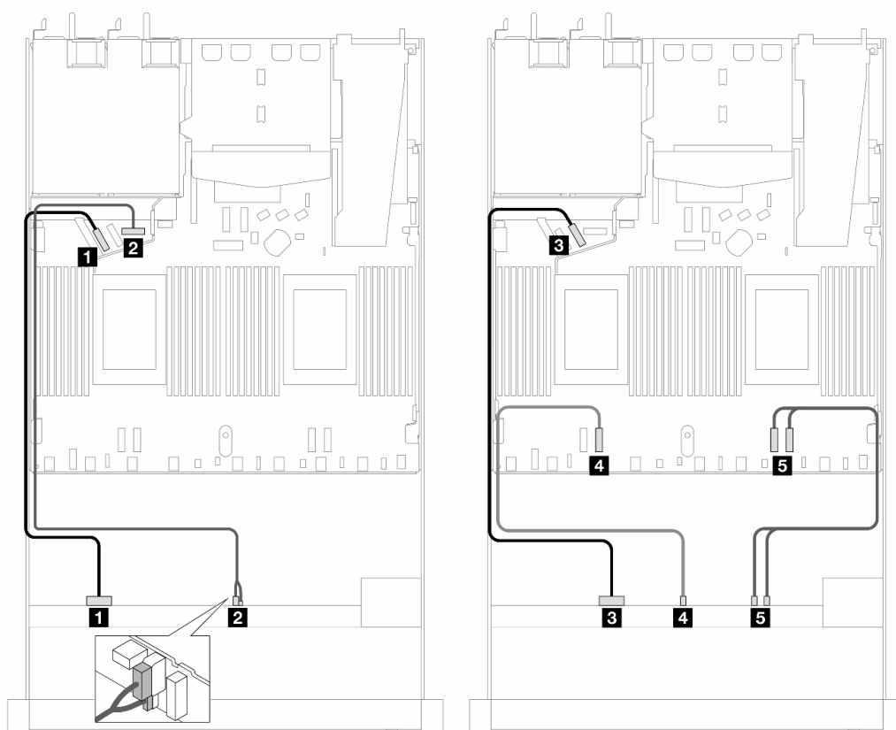
圖例 350. 用於液冷的 10 個 NVMe 磁碟機 ( Gen 5 背板 ) 的機載佈線
