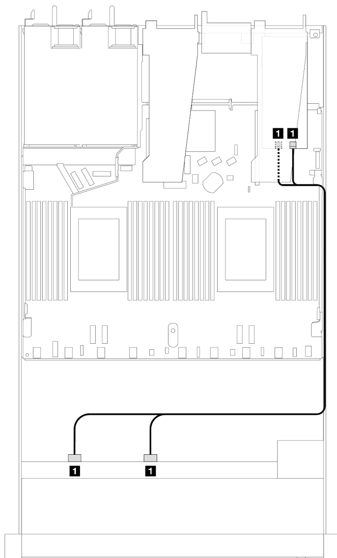
圖例 343. 包含 8i 或 16i SFF RAID 配接卡 (Gen 3) 的 8 x 2.5 吋前方 SAS/SATA 機槽的纜線佈線
