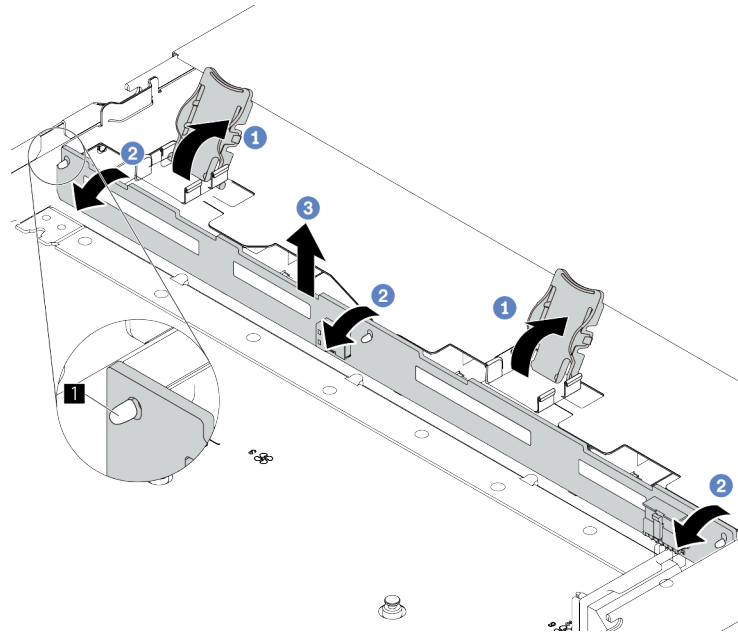
圖例 15. 卸下 3.5 吋硬碟背板
