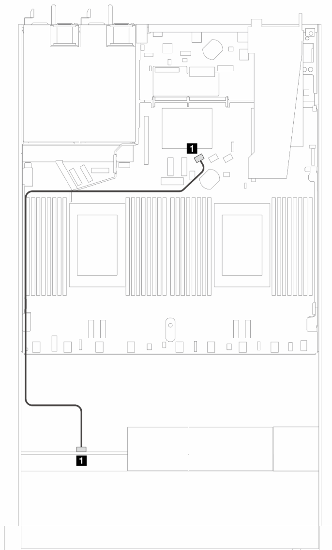
圖例 407. 4 x 2.5 吋前方 SAS/SATA 硬碟機載配置的纜線佈線
