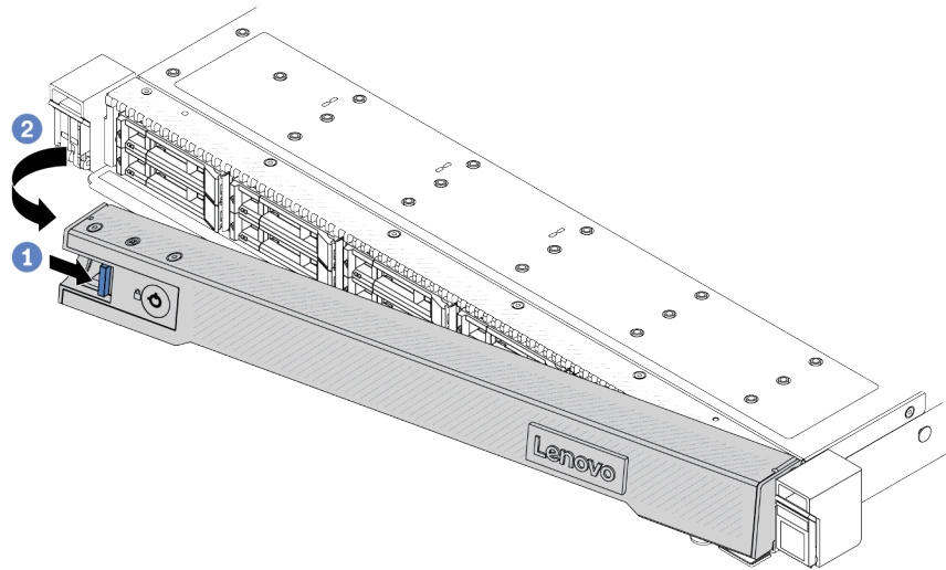
圖例 257. 卸下安全擋板
