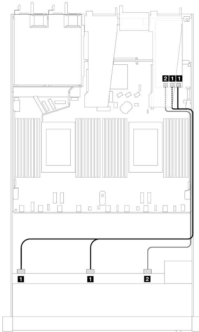
圖例 391. 包含 16i SFF RAID 配接卡 (Gen 3) 的 10 個前方 SAS/SATA 機槽的纜線佈線
