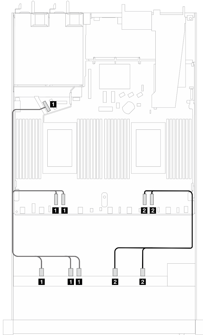
圖例 456. 10 x 2.5 NVMe 前方硬碟機載配置的纜線佈線
