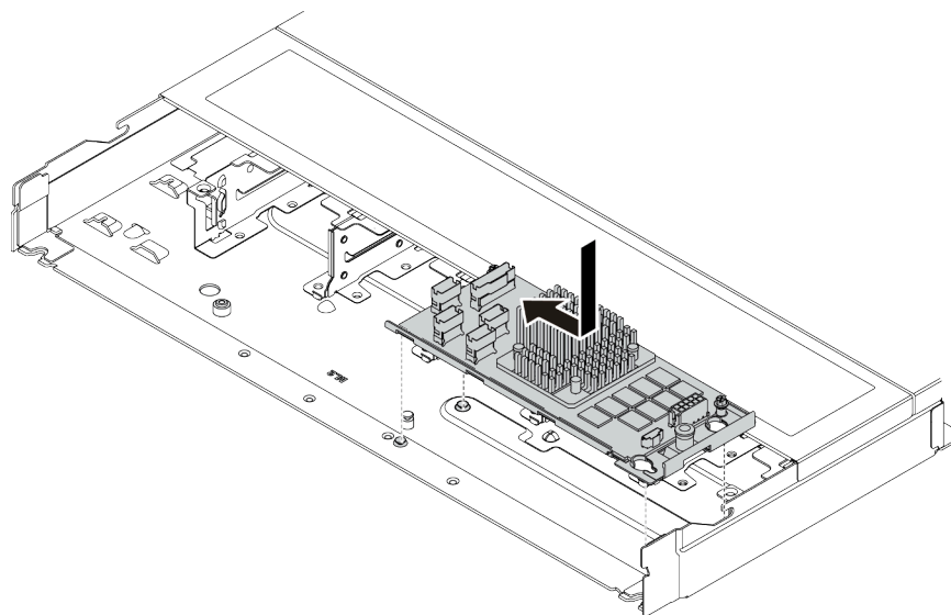
圖例 89. 安裝內部 CFF RAID 配接卡
