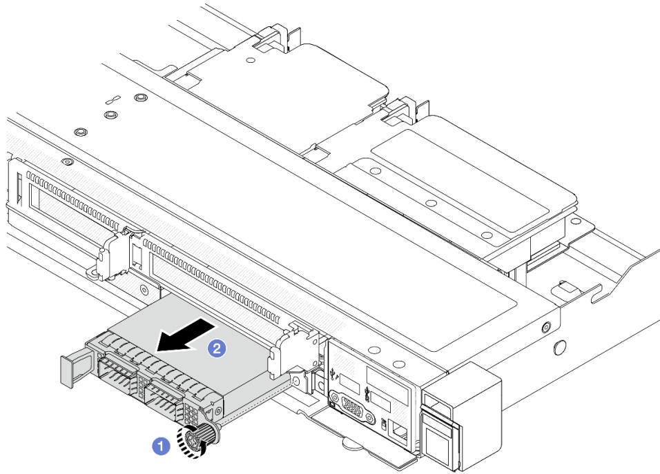
圖例 48. 卸下正面 OCP 模組
