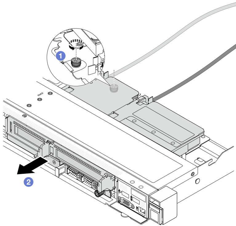
圖例 38. 卸下正面擴充卡匣
