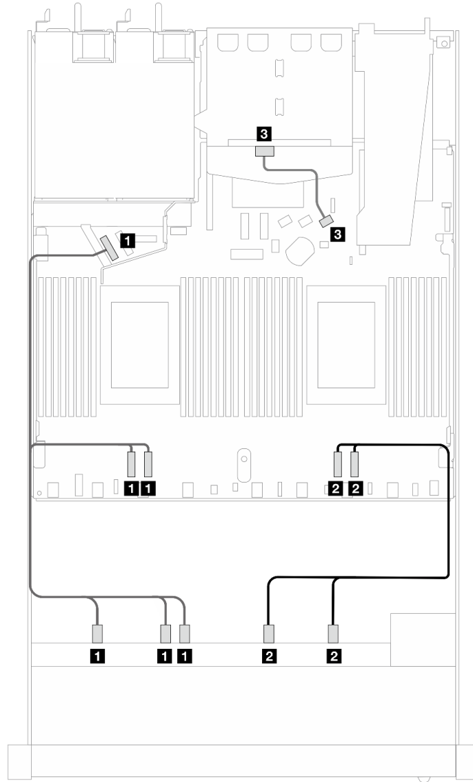
圖例 457. 安裝 2 x 2.5 後方 SAS/SATA 硬碟之 10 x 2.5 NVMe 前方硬碟機載配置的纜線佈線
