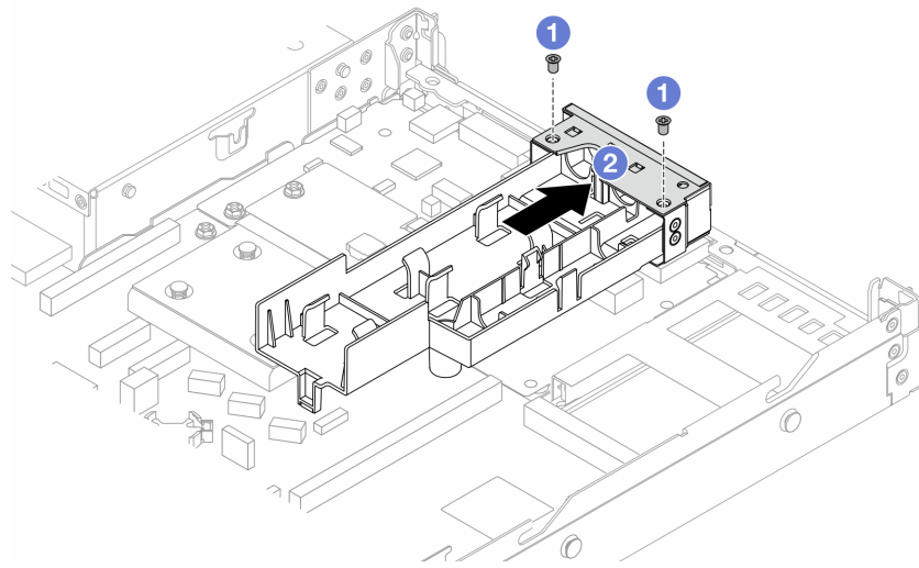
圖例 96. 卸下固定器蓋
