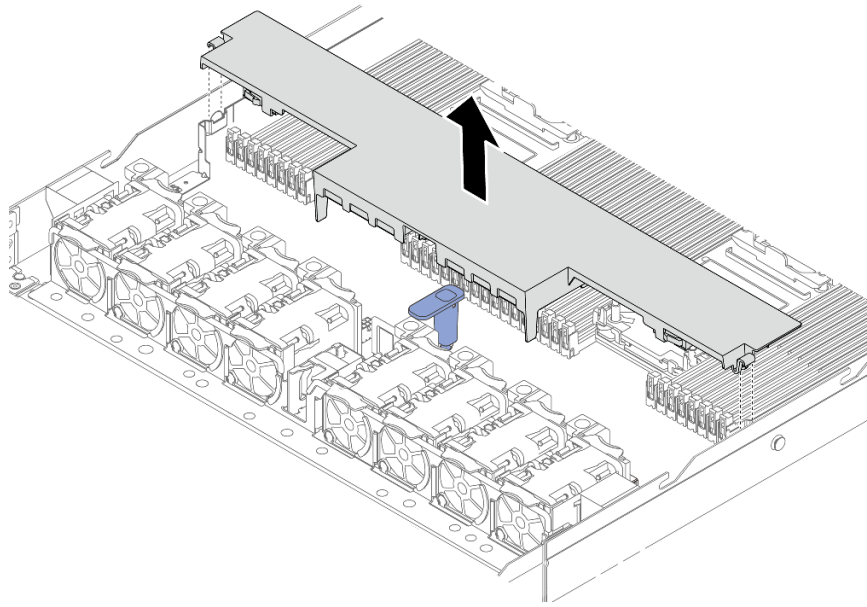
圖例 11. 卸下空氣擋板
