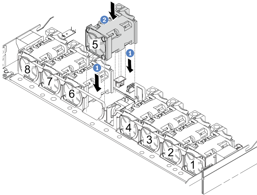
圖例 278. 安裝系統風扇
