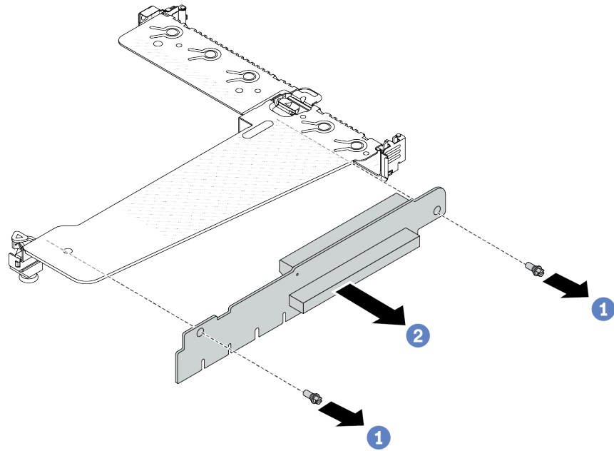
圖例 252. 卸下擴充卡
