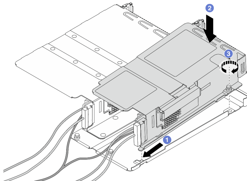
圖例 47. 組裝兩個擴充卡匣
