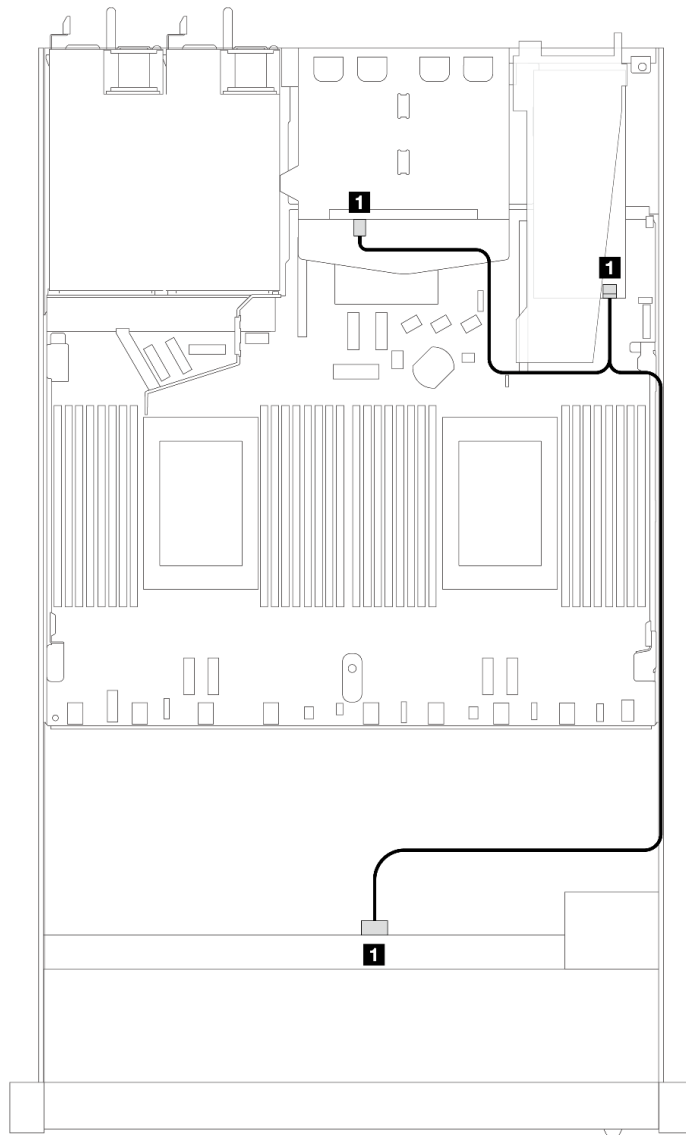
圖例 401. 配備 8i SFF RAID 配接卡 (Gen 4) 和後方 2 x 2.5 吋 SAS/SATA 硬碟之 4 x 3.5 吋前方 SAS/SATA 機槽的纜線佈線
