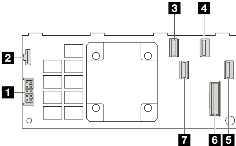
圖例 300. Gen 4 16i CFF RAID 配接卡 ( 四個埠接頭 )
