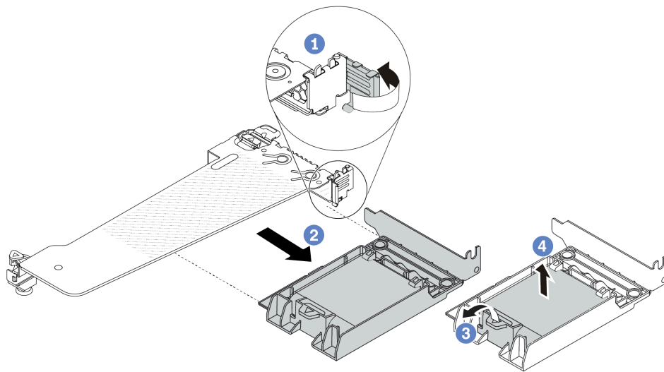
圖例 201. 從擴充卡上卸下 RAID 超級電容器組件
