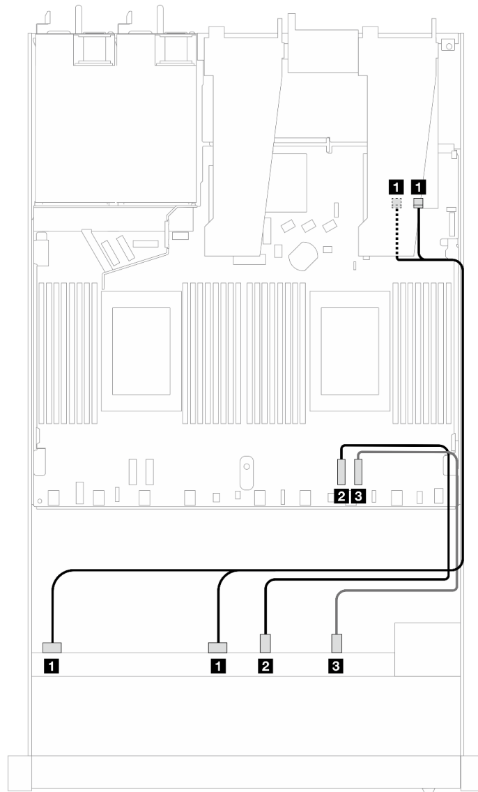
圖例 340. 包含 8i 或 16i SFF RAID 配接卡 (Gen 3) 的 6 個 SAS/SATA 硬碟和 2 個 AnyBay 硬碟和 2 個 NVMe 前方機槽的纜線佈線
