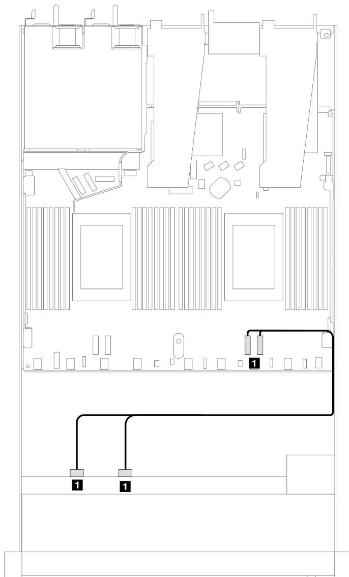
圖例 365. 包含一個處理器的 4 x 2.5 吋前方 NVMe 機槽機載配置的纜線佈線
