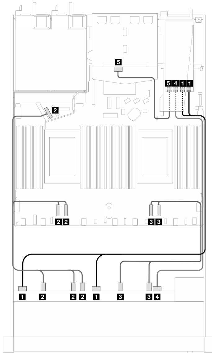
圖例 455. 包含 16i SFF RAID 配接卡 (Gen 3) 的 10 個前方 AnyBay 硬碟和 2 個後方 SAS/SATA 硬碟的纜線佈線
