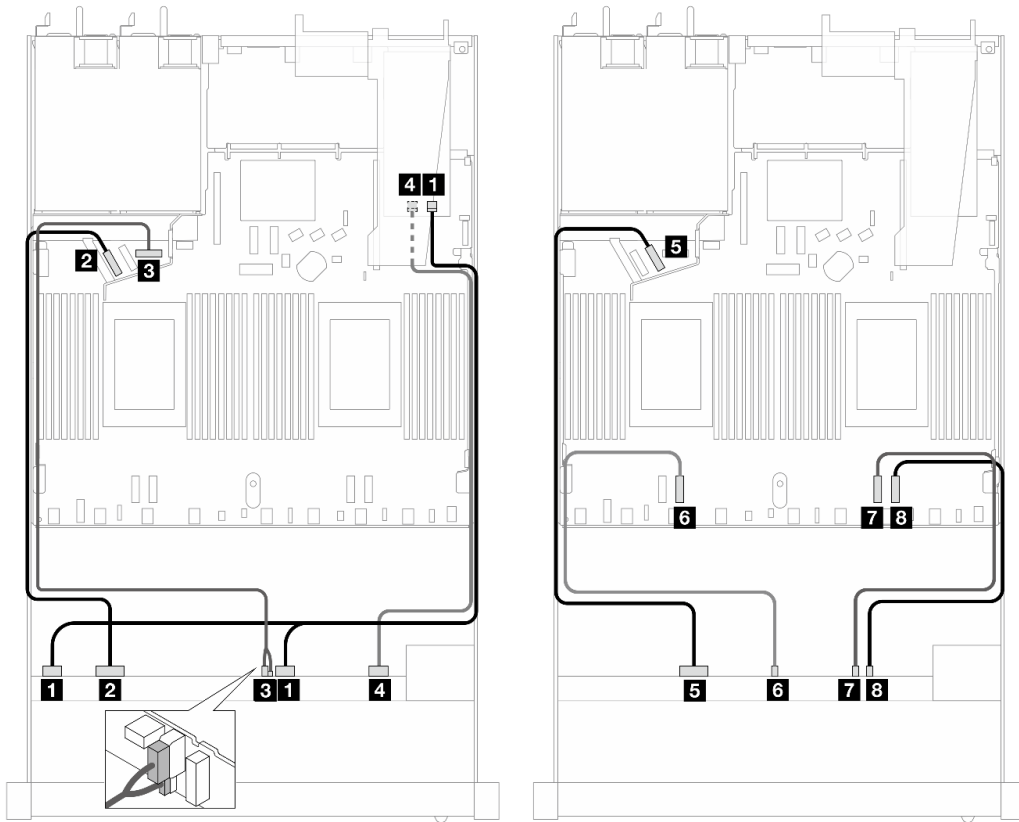
圖例 470. 包含 16i SFF RAID 配接卡 (Gen 4) 的 10 個前方 AnyBay 硬碟的纜線佈線
