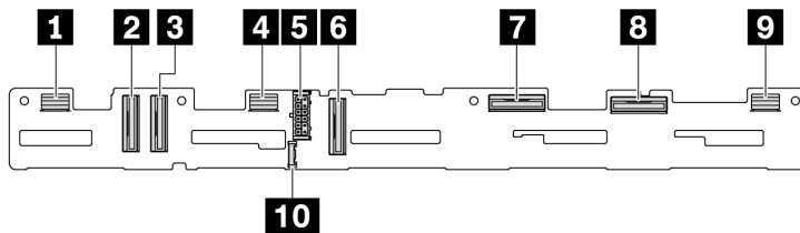
圖例 284. 10 x 2.5 吋 AnyBay 背板
