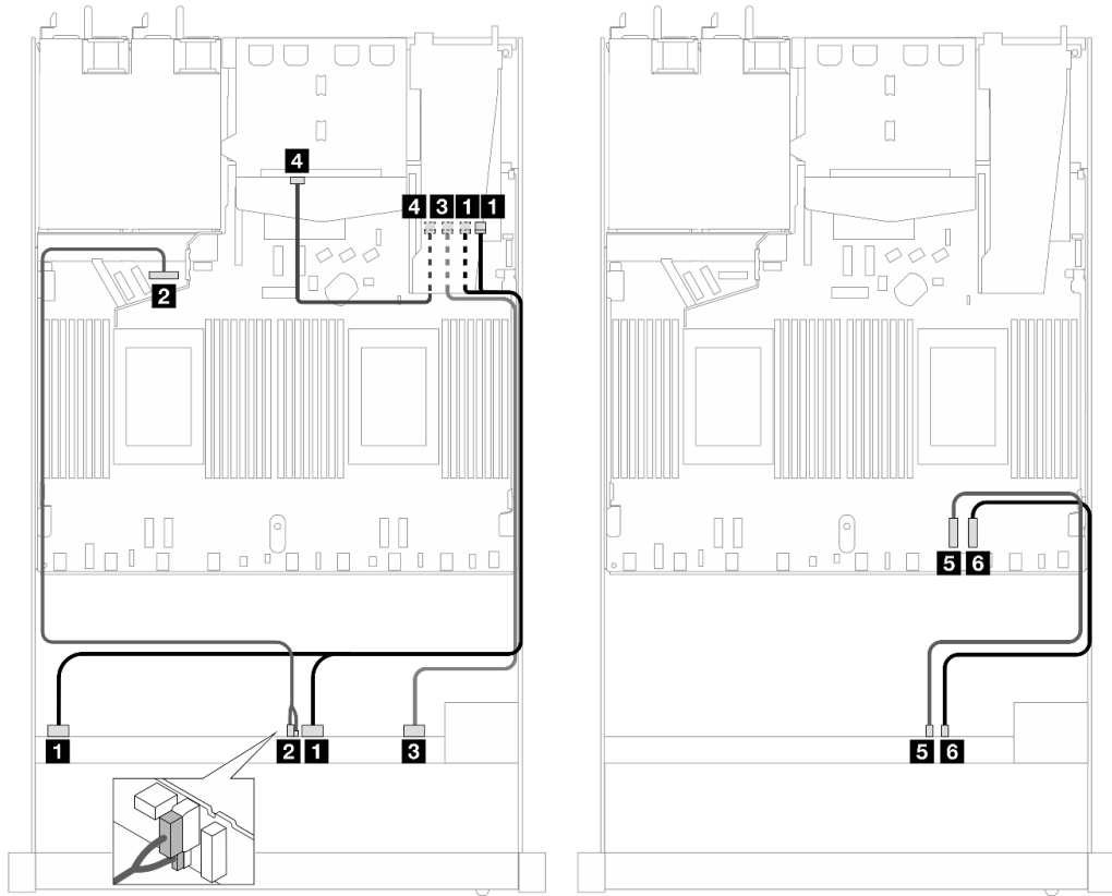
圖例 462. 六個前方 SAS/SATA 硬碟和四個前方 AnyBay 機槽以及 16i SFF RAID 配接卡 (Gen 3) (已安裝兩個後方 SAS/SATA 硬碟) 的纜線佈線
