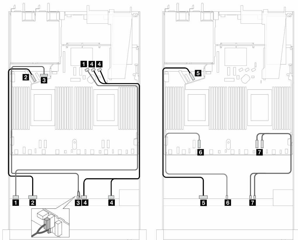
圖例 351. 10 個 AnyBay 前方硬碟 ( Gen 5 背板 ) 配置的纜線佈線
