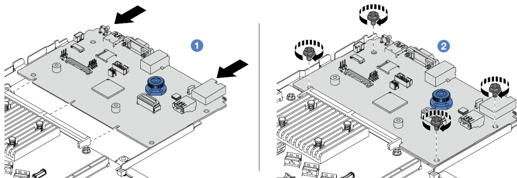
圖例 271. 安裝系統 I/O 板
