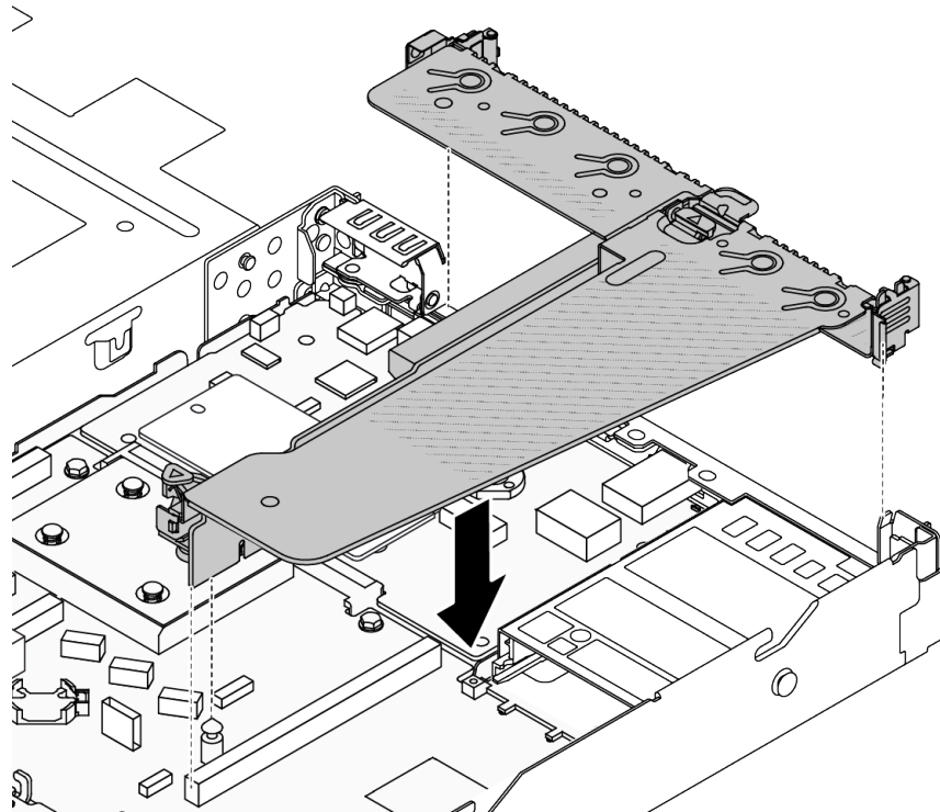
圖例 255. 安裝擴充卡組件
