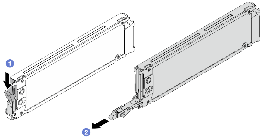
圖例 78. 卸下 EDSFF 硬碟
