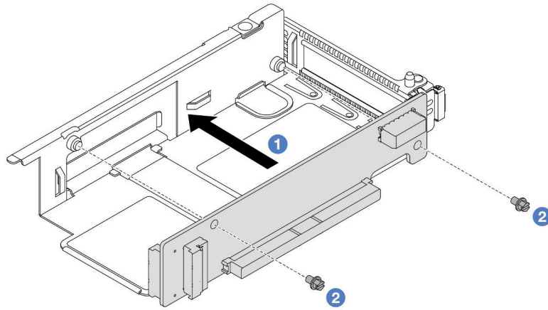
圖例 44. 將擴充卡安裝到半高匣
