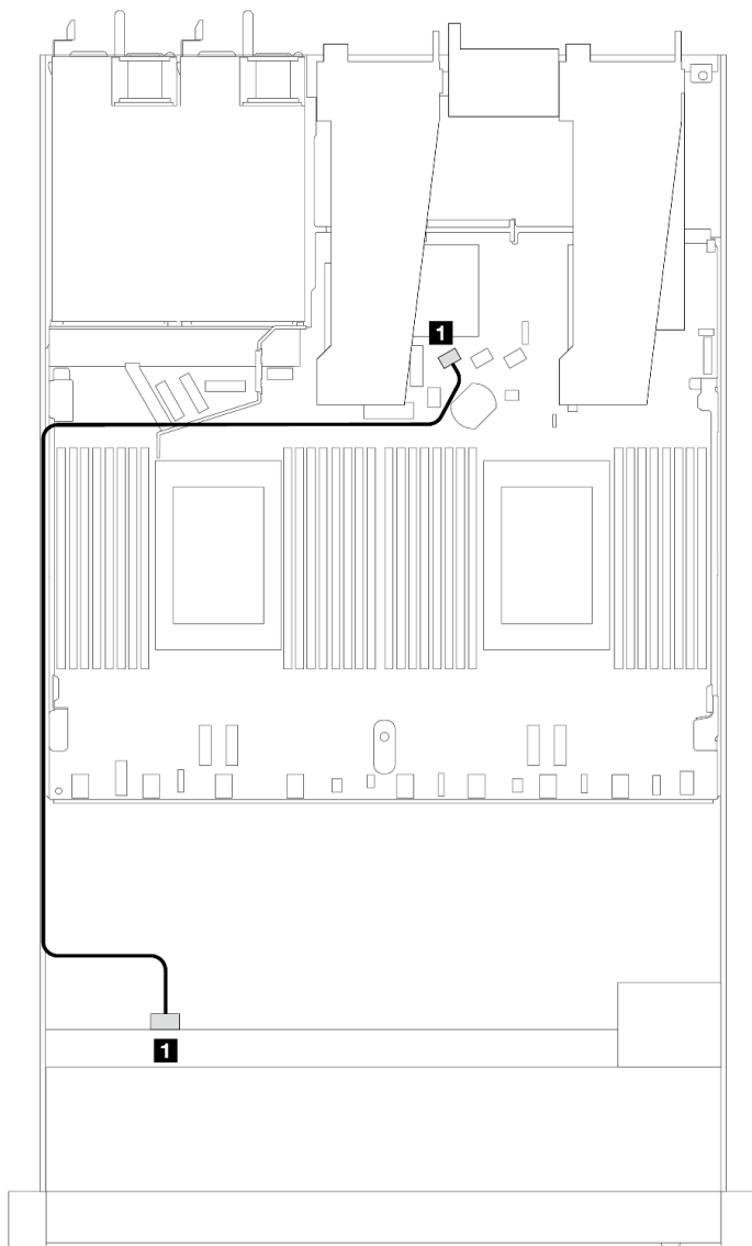
圖例 362. 4 x 2.5 吋前方 AnyBay 機槽機載配置的纜線佈線
