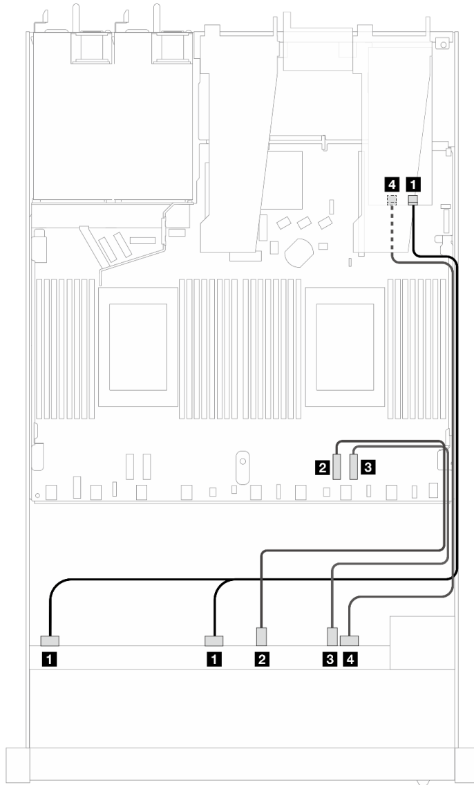
圖例 335. 包含 8i 或 16i SFF RAID 配接卡 (Gen 4) 的六個前方 SAS/SATA 硬碟和四個前方 AnyBay 機槽的纜線佈線
