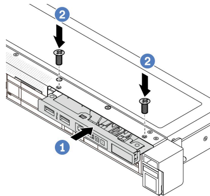
圖例 57. 將正面 I/O 模組安裝在 3.5 吋機箱上
