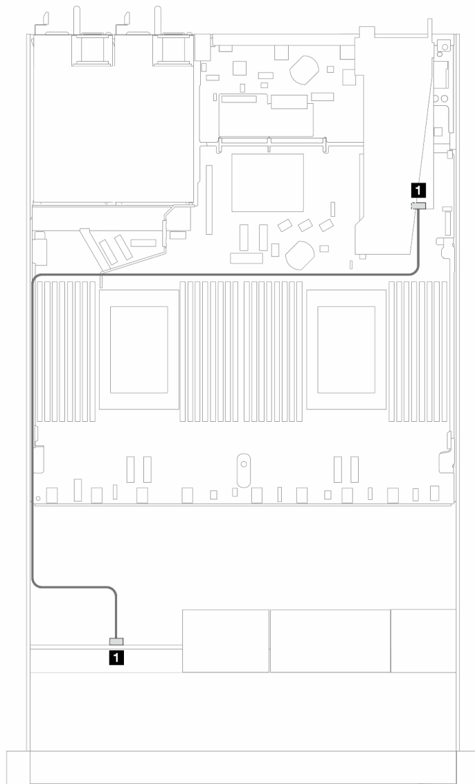
圖例 409. 包含 8i SFF RAID 配接卡 (Gen 3/4) 的 4 x 2.5 吋前方 SAS/SATA 機槽的纜線佈線
