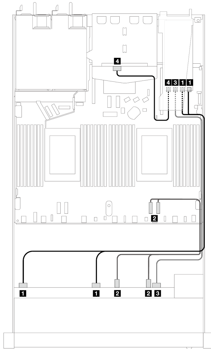
圖例 438. 6 個前方 SAS/SATA 硬碟和 4 個前方 AnyBay 機槽以及 16i SFF RAID 配接卡 (Gen 3) (已安裝 2 x 2.5 後方 SAS/SATA 硬碟) 的纜線佈線
