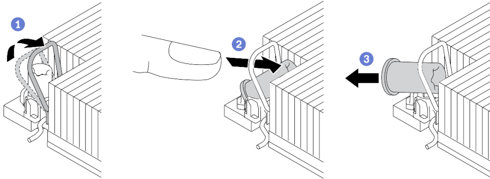
圖例 71. 從散熱槽卸下 Torx T30 螺帽
