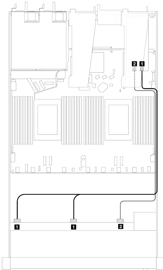
圖例 347. 包含 16i SFF RAID 配接卡 (Gen 4) 的 10 個前方 SAS/SATA 硬碟的纜線佈線
