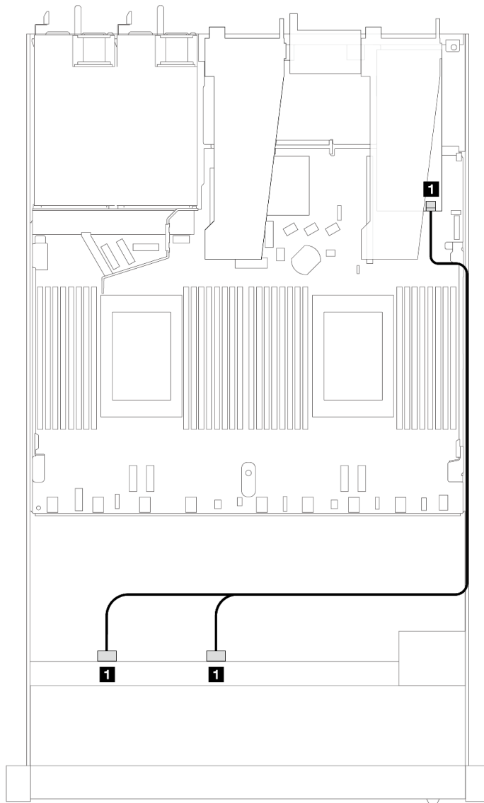
圖例 370. 包含 8i 或 16i SFF RAID 配接卡 (Gen 4) 的 8 x 2.5 吋前方 SAS/SATA 機槽的纜線佈線
