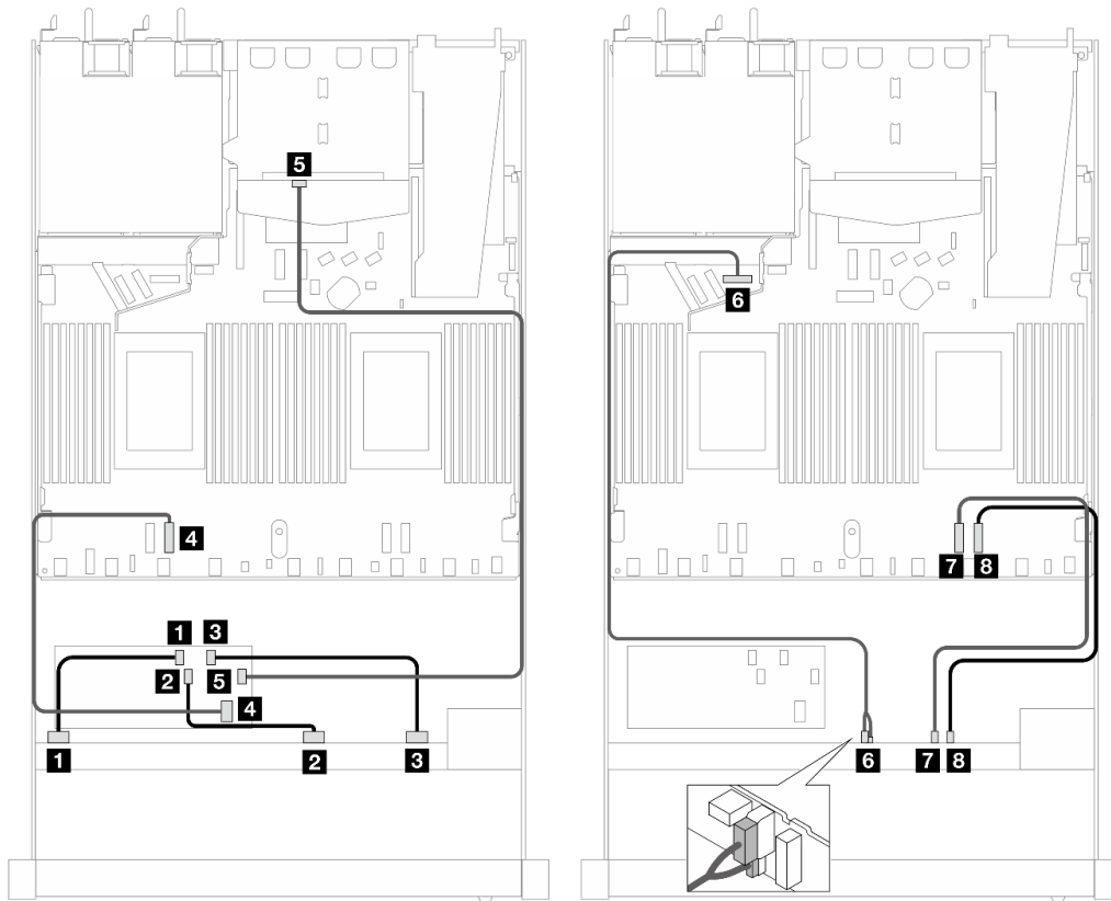
圖例 464. 六個前方 SAS/SATA 和四個前方 AnyBay 硬碟以及 16i CFF HBA/RAID 配接卡 (Gen 4) 和安裝兩個後方 SAS/SATA 硬碟的纜線佈線
