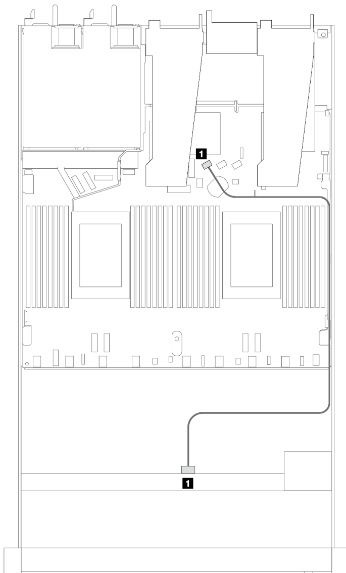
圖例 357. 4 x 3.5 吋前方 SAS/SATA 機槽機載配置的纜線佈線
