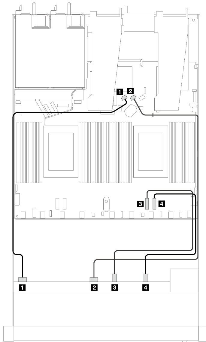
圖例 332. 六個 SAS/SATA 和四個 NVMe 前方硬碟機載配置的纜線佈線
