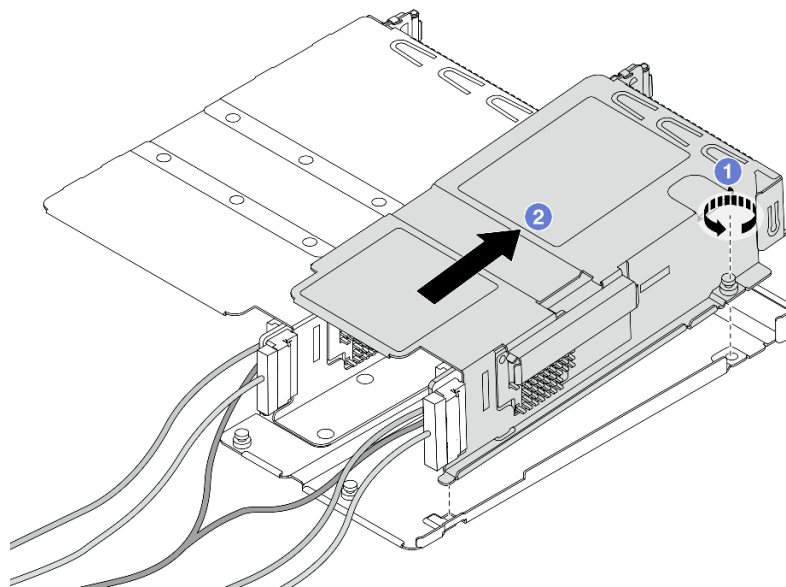
圖例 40. 將兩個匣分開
