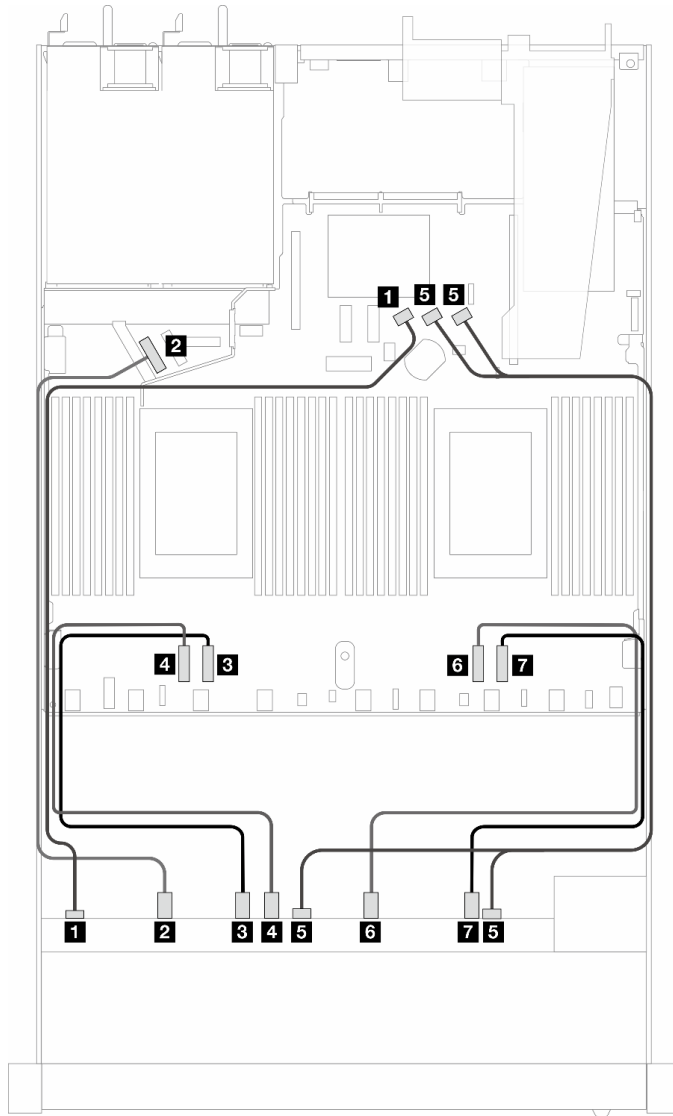
圖例 354. 10 個 AnyBay 前方硬碟 ( Gen 4 背板 ) 配置的纜線佈線
