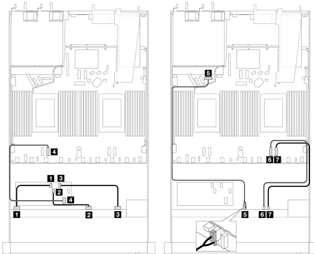
圖例 463. 包含 16i HBA/RAID 配接卡 (Gen 4) 的六個前方 SAS/SATA 硬碟和四個前方 AnyBay 機槽的纜線佈線
