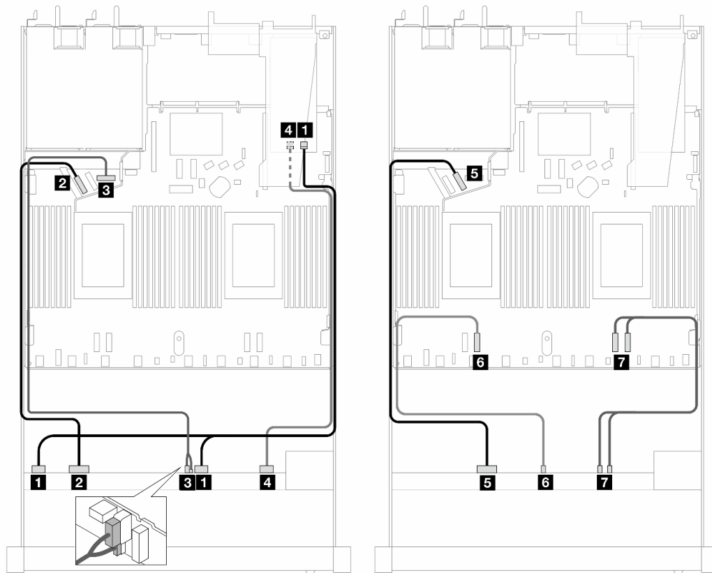
圖例 352. 包含 16i SFF RAID 配接卡 (Gen 4) 的 10 個前方 AnyBay 硬碟的纜線佈線
