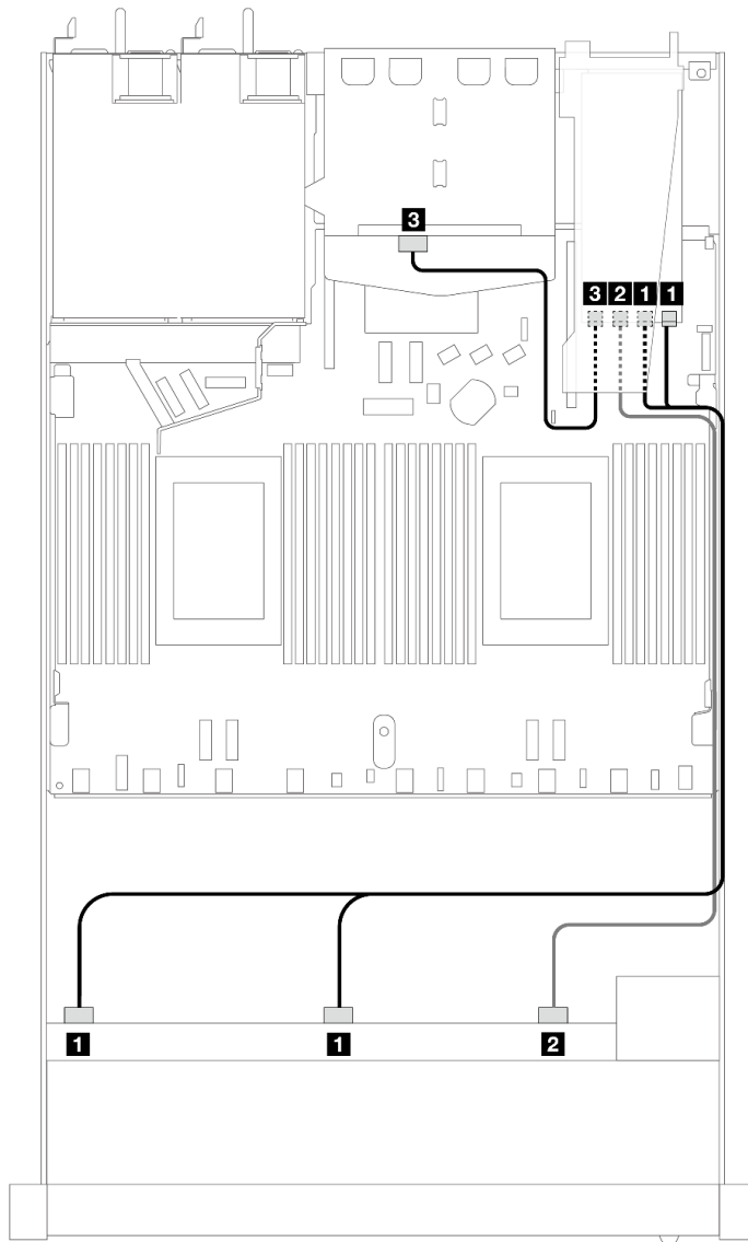
圖例 449. 安裝 2 x 2.5 後方 SAS/SATA 硬碟之 10 個前方 SAS/SATA 機槽和 16i SFF RAID 配接卡 (Gen 3) 的纜線佈線
