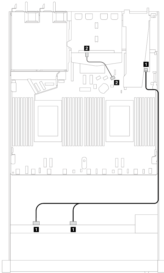
圖例 372. 配備 8i SFF RAID 配接卡 (Gen 4) (已安裝 2 x 2.5 SAS/SATA 背面硬碟) 之 8 x 2.5 吋前方 SAS/SATA 機槽的纜線佈線
