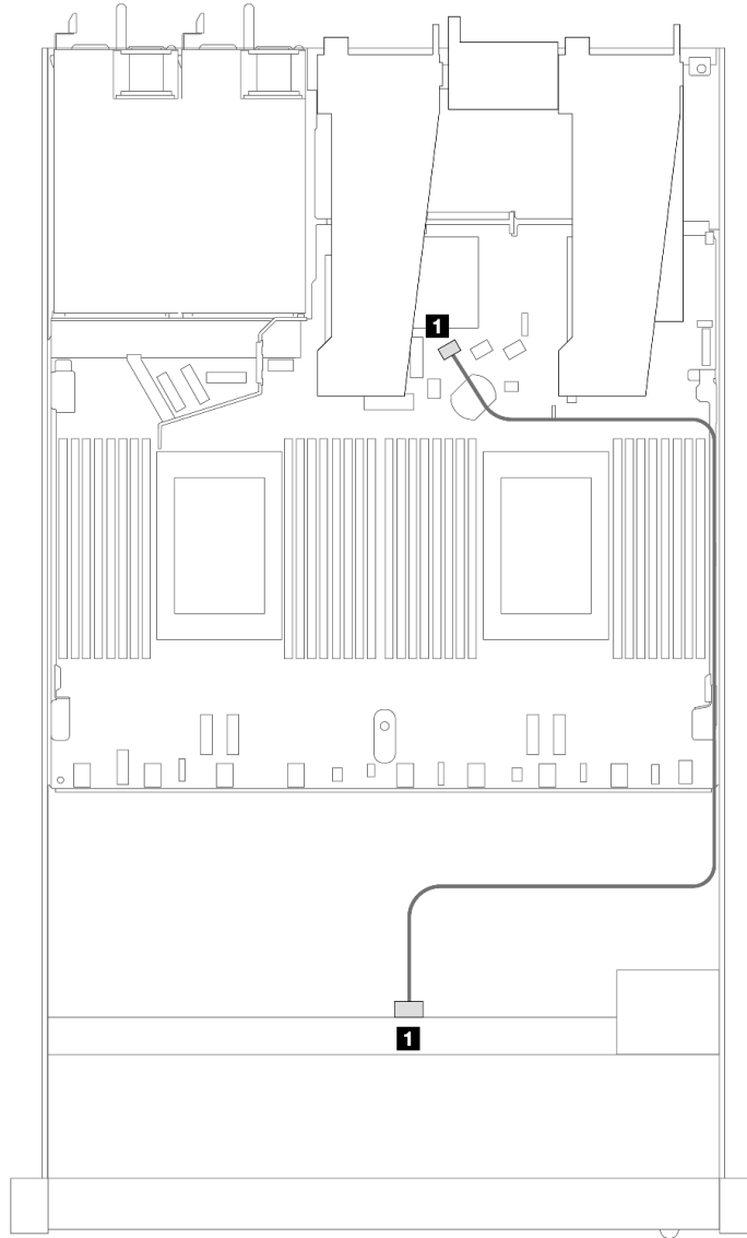
圖例 395. 4 x 3.5 吋前方 SAS/SATA 機槽機載配置的纜線佈線
