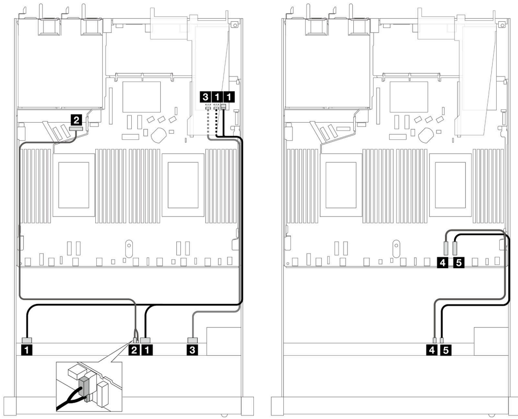
圖例 461. 包含 16i SFF RAID 配接卡 (Gen 3) 的六個前方 SAS/SATA 硬碟和四個前方 AnyBay 機槽的纜線佈線
