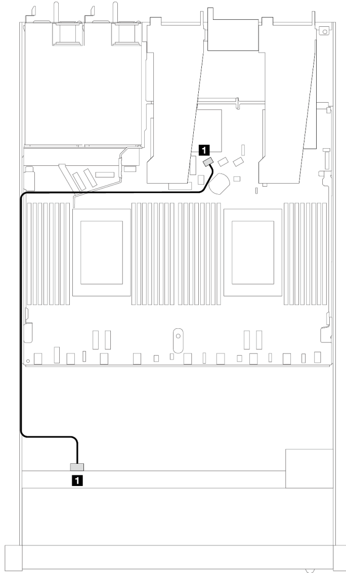
圖例 402. 4 x 2.5 吋前方 AnyBay 機槽機載配置的纜線佈線
