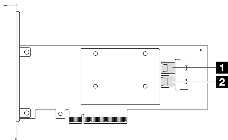
圖例 296. Gen 3 8i SFF RAID/HBA 配接卡 ( 兩個埠接頭 )
