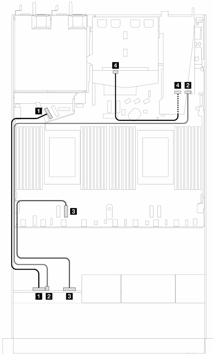
圖例 419. 包含 8i SFF RAID 配接卡 (Gen 3) 和 2 x 2.5 吋後方 SAS/SATA 硬碟的 4 x 2.5 吋前方 AnyBay 機槽的纜線佈線
