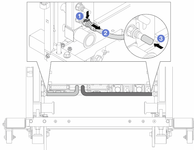
圖例 114. 移除 quick connect 插頭
