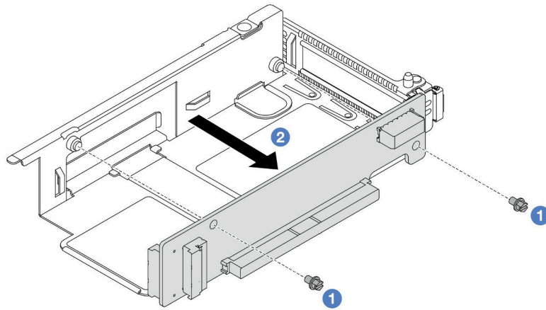
圖例 42. 從半高匣卸下擴充卡
