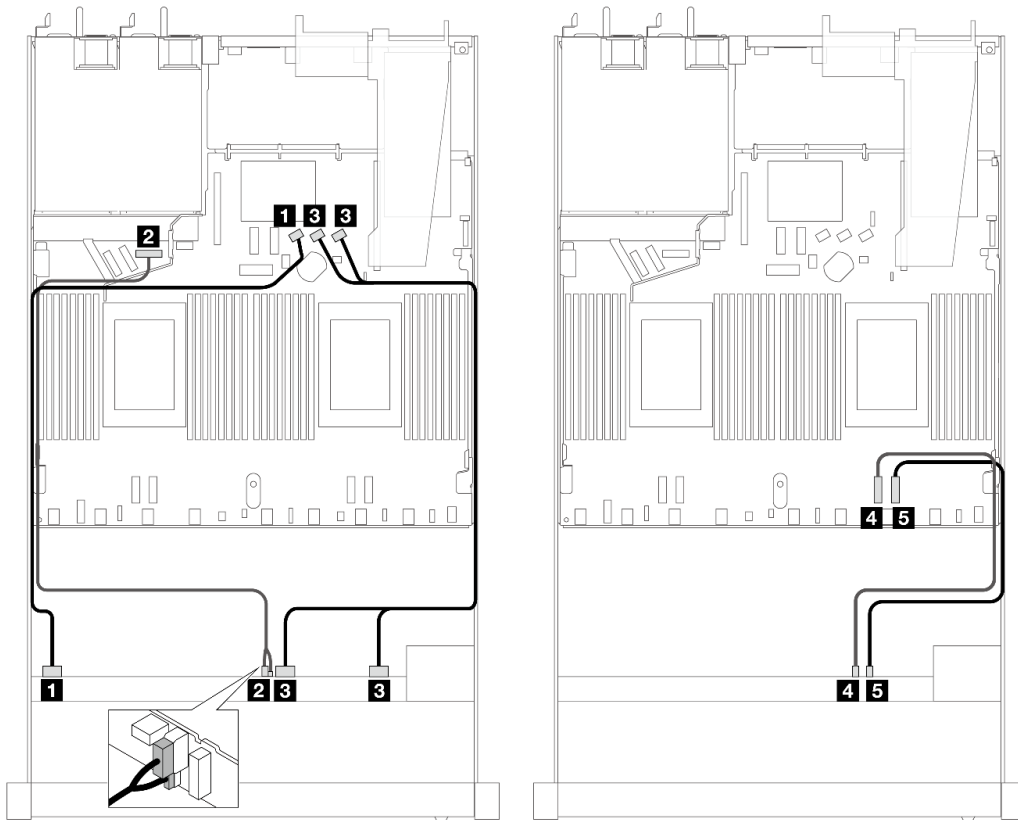
圖例 458. 6 x 2.5 吋 SAS/SATA 前方硬碟和 4 x 2.5 吋 AnyBay 前方硬碟之機載配置的纜線佈線
