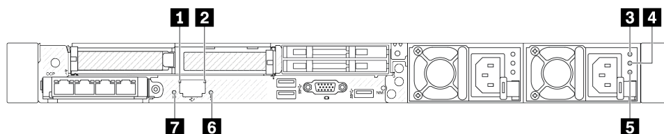
圖例 22. 背面 LED 概觀
