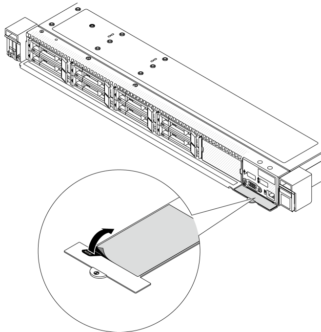
圖例 28. 拉出式資訊標籤上的 Lenovo XClarity Controller 網路存取標籤
