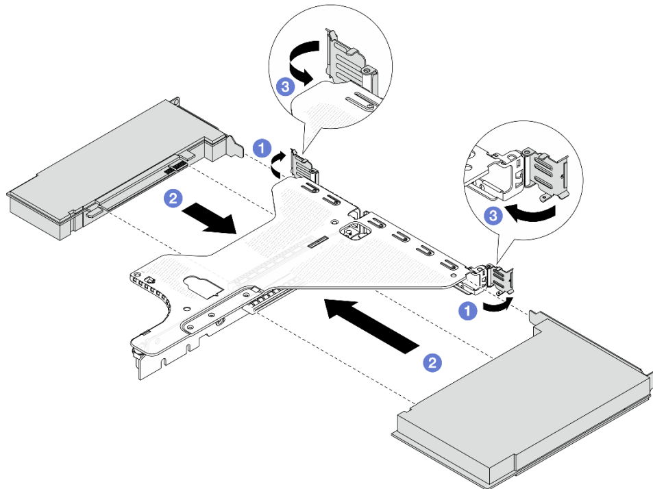
Figura 186. Instalación del adaptador PCIe en el conjunto de expansión LP-FH
