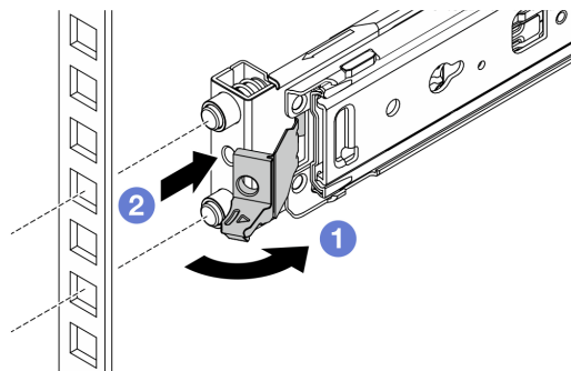
Figura 29. Extracción del riel en la parte frontal
