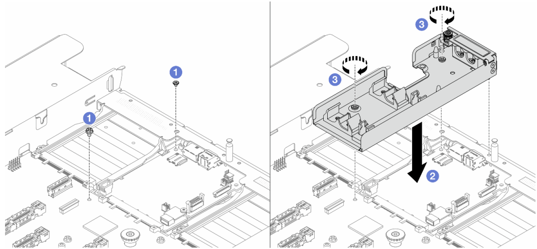
Figura 123. Instalación del soporte de manguera
