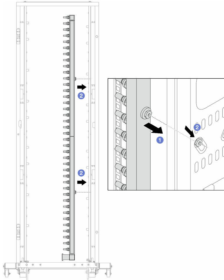
Figura 170. Instalación del múltiple
