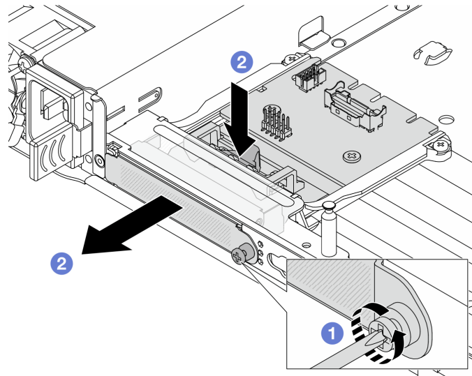
Figura 85. Extracción de la tarjeta de interposición de OCP trasera
