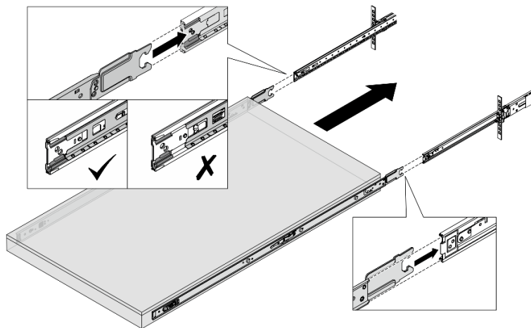
Figura 52. Interbloqueo de rieles
