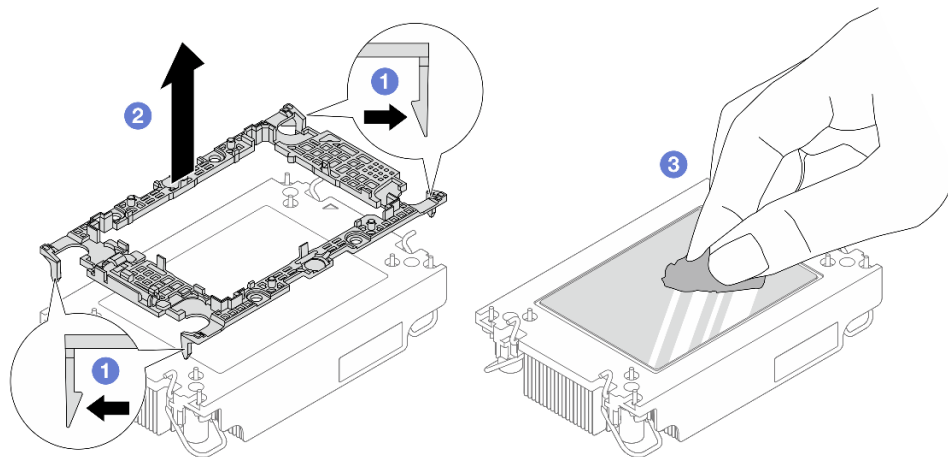
Figura 191. Separación de un transportador de procesador del disipador de calor
