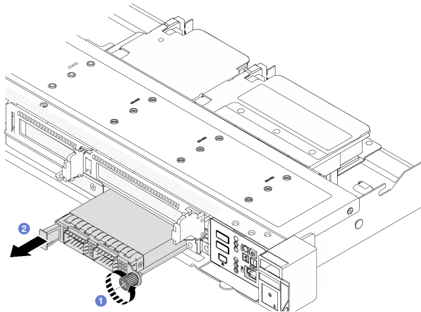
Figura 81. Extracción del módulo de OCP frontal
