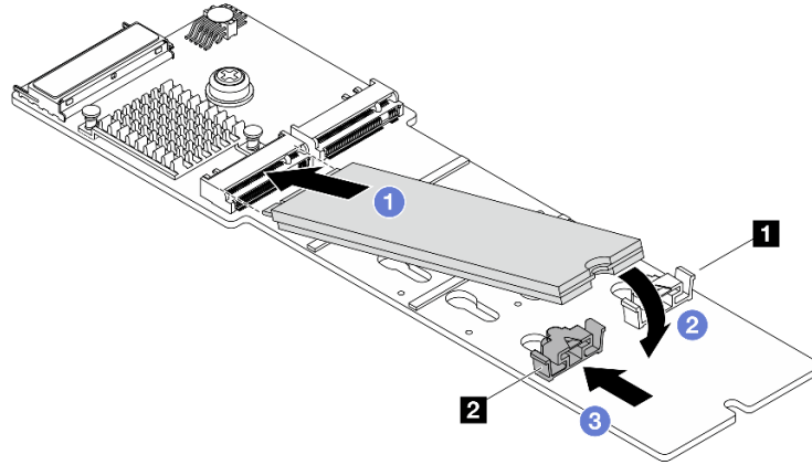
Figura 107. Instalación de la unidad M.2
