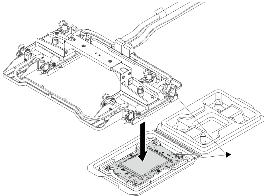
Figura 125. Instalación de un procesador
