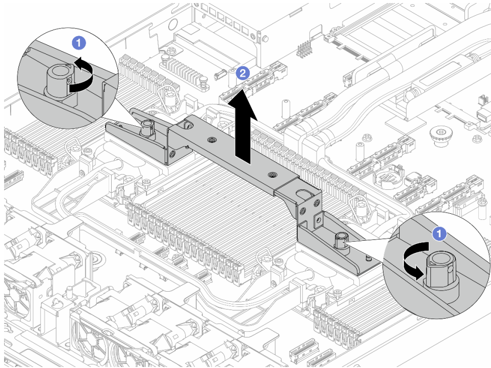
Figura 128. Extracción del asa del módulo
