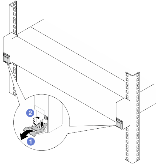
Figura 35. Soltar los tornillos de los pestillos del bastidor
