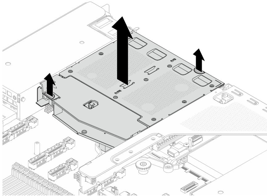
Figura 201. Extracción del compartimiento de la unidad trasera de 2,5"
