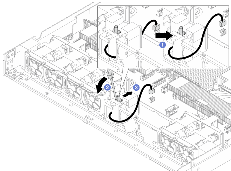
Figura 110. Extracción del conmutador de intrusión
