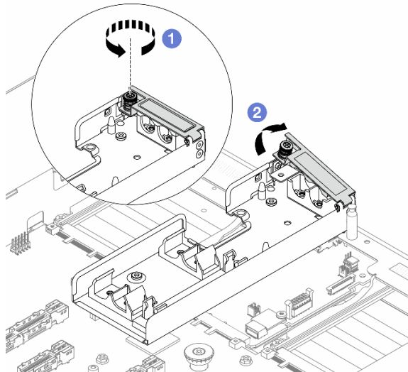
Figura 124. Apertura de la cubierta del soporte
