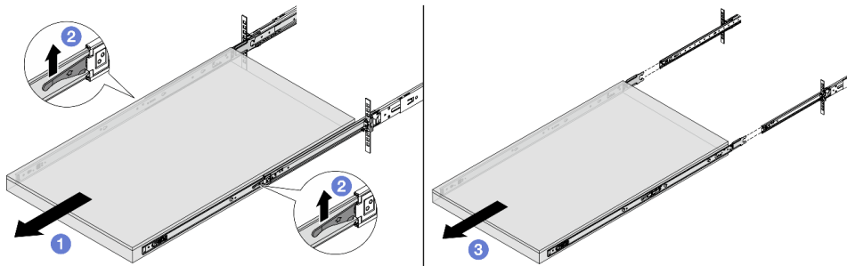
Figura 47. Extracción del servidor
