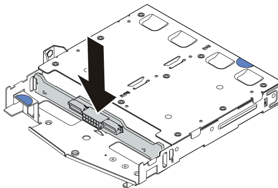
Figura 62. Instalación de la placa posterior
