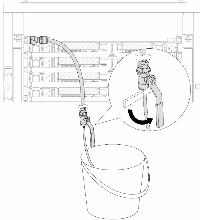
Figura 175. Apertura de la válvula de purga del lado de suministro
