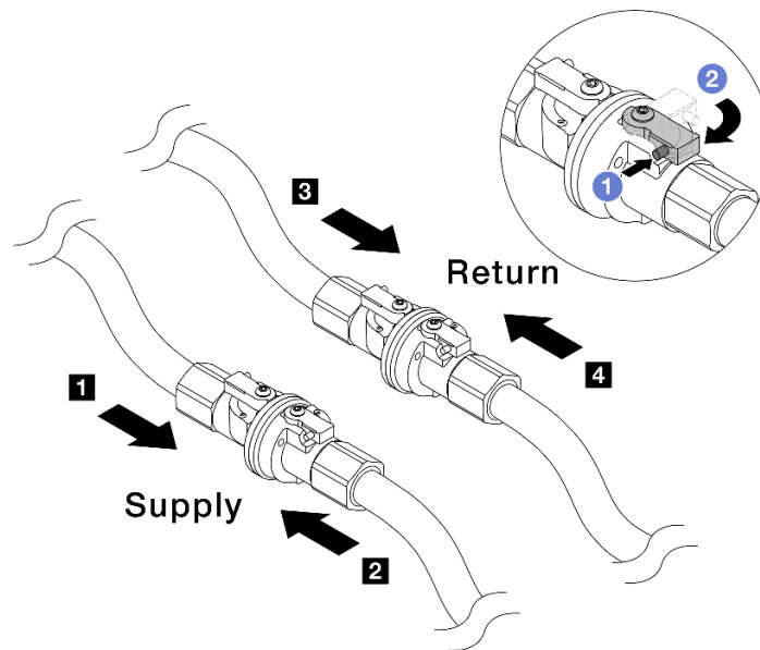
Figura 180. Apertura de las válvulas de bola
