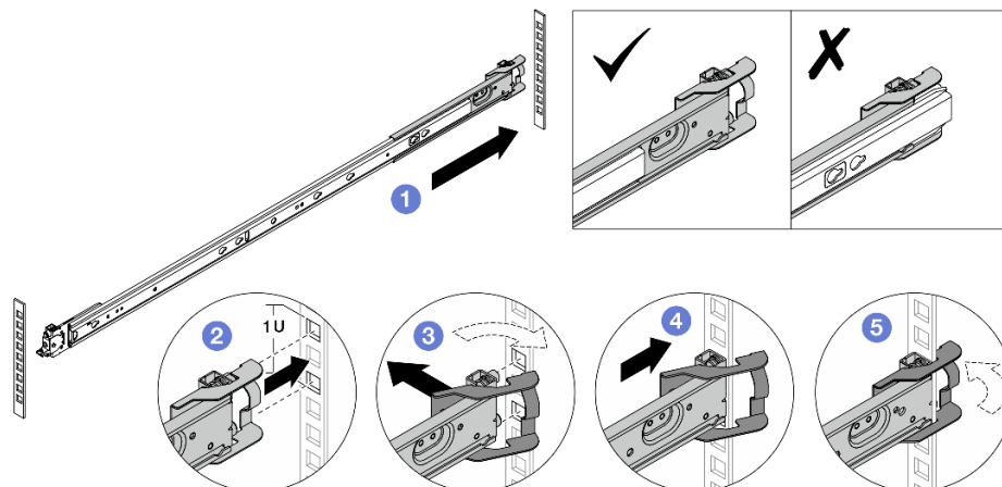
Figura 31. Instalación de las patillas de montaje posteriores
