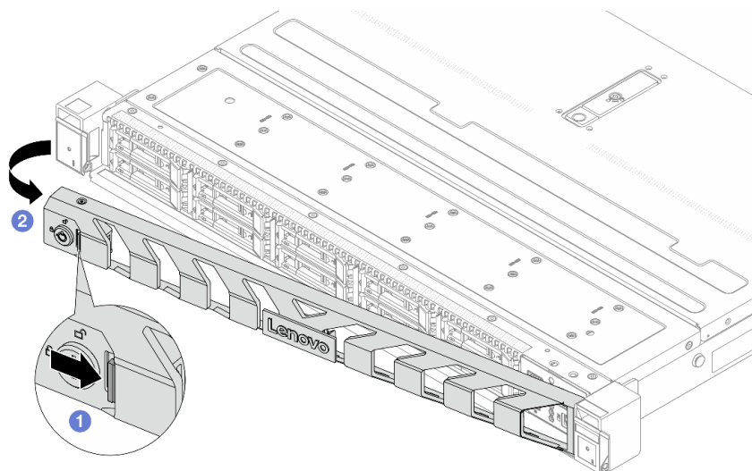
Figura 266. Extracción del marco biselado de seguridad
