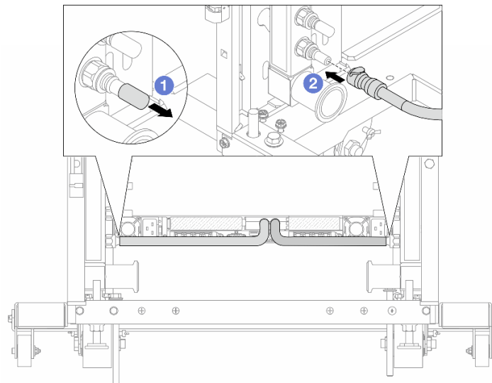
Figura 155. Instalación del conector rápido
