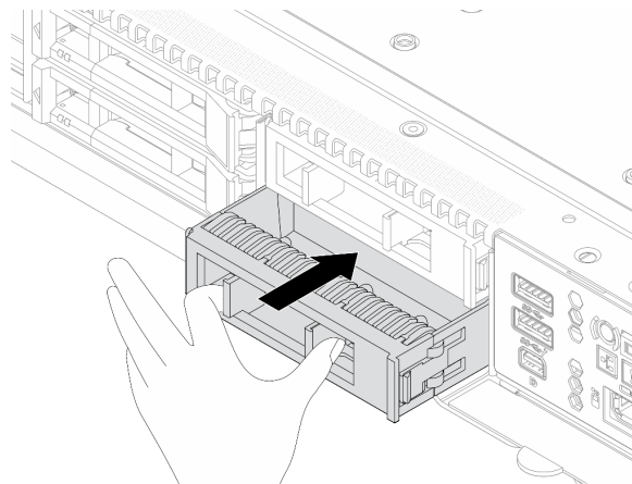
Figura 92. Instalación de un relleno de unidad
