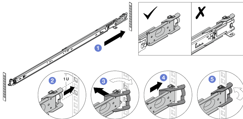
Figura 33. Instalación de las patillas de montaje posteriores
