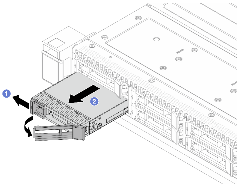
Figura 91. Extracción de una unidad de intercambio en caliente
