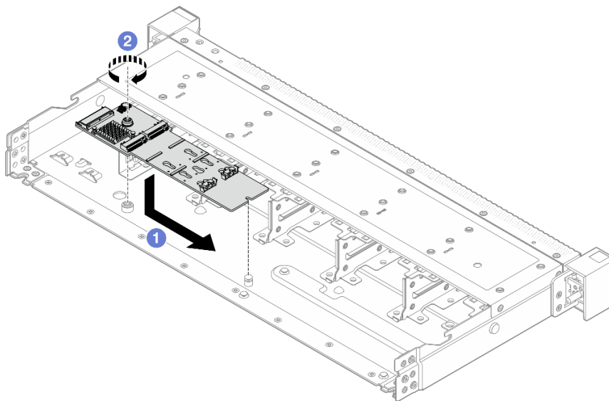
Figura 106. Instalación de la placa posterior de M.2
