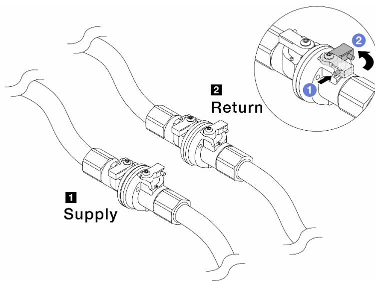
Figura 162. Cierre de las válvulas de bola
