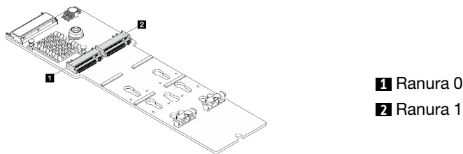
Figura 105. Ranura de unidad M.2
