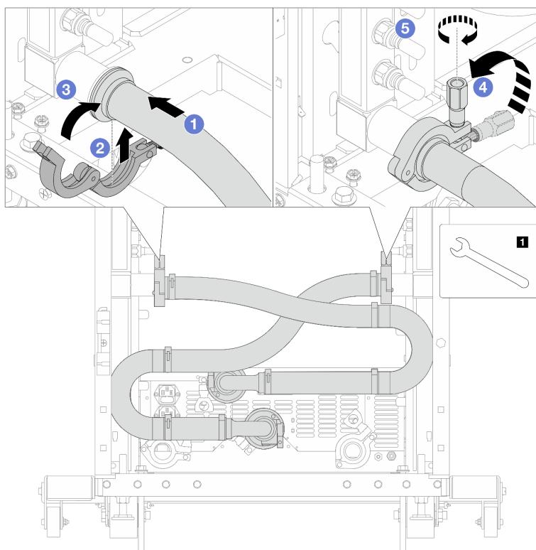
Figura 151. Instalación de conjunto de conexión
