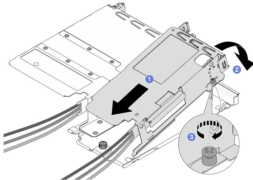
Figura 80. Montaje de los dos compartimientos de expansión
