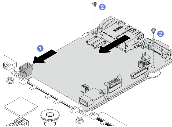
Figura 278. Instalación de la placa de E/S del sistema
