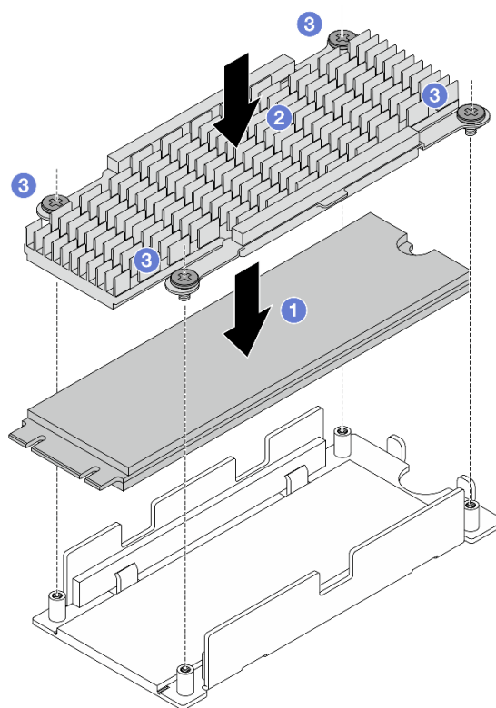
Figura 212. Instalación de una unidad M.2
