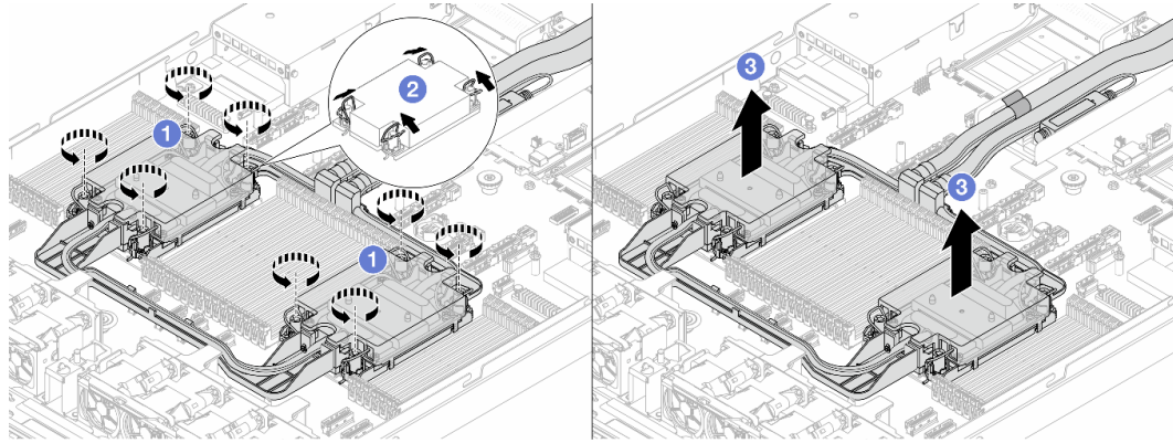
Figura 121. Extracción del Módulo NeptCore
