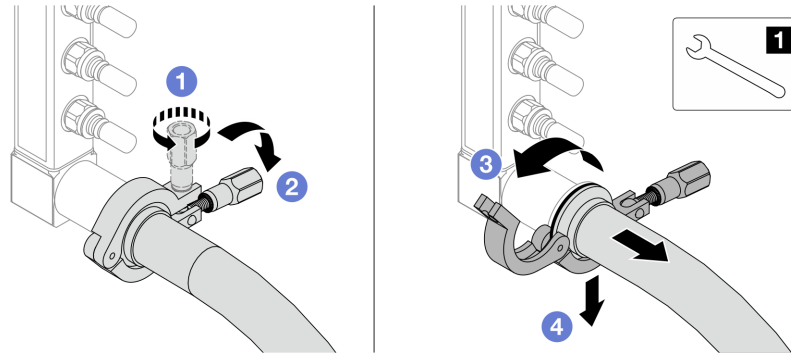
Figura 147. Separación del múltiple del juego de conexión
