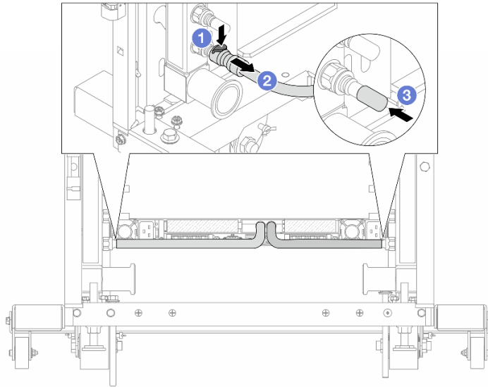
Figura 140. Extracción de los conectores rápidos
