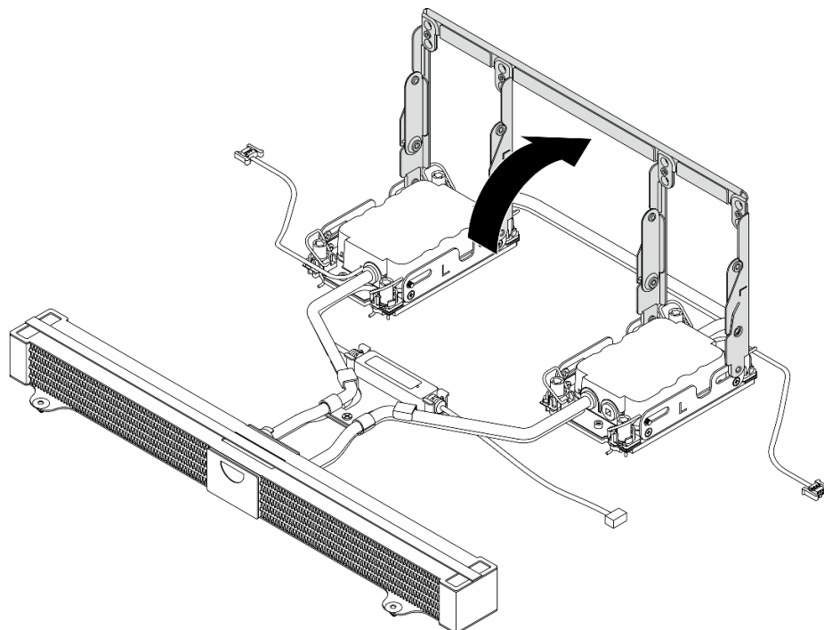
Figura 118. Apertura del asa
