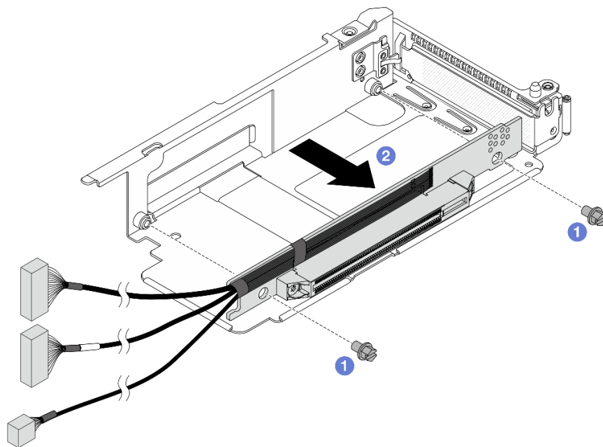
Figura 75. Extracción de la tarjeta de expansión del compartimiento de bajo perfil
