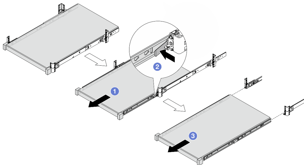
Figura 37. Extracción del servidor
