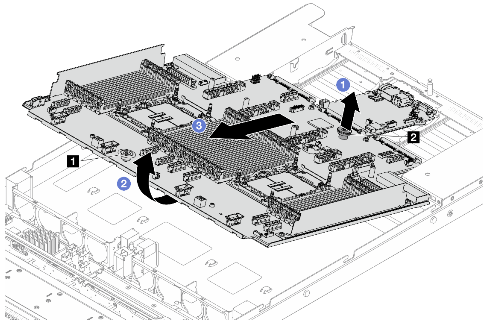
Figura 279. Extracción del conjunto de la placa del sistema
