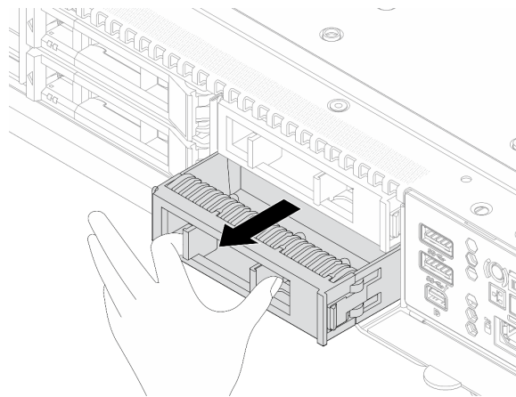
Figura 93. Extracción de un relleno de unidad
