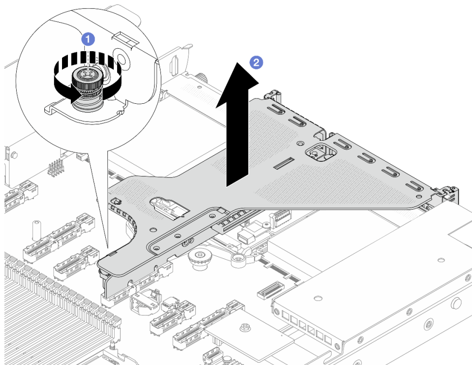
Figura 261. Extracción del conjunto de expansión
