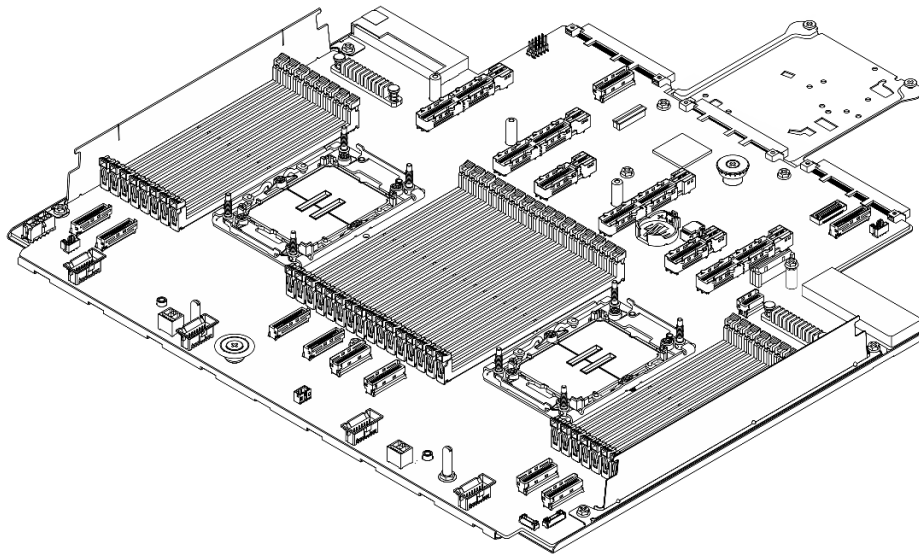
Figura 281. La placa del procesador
