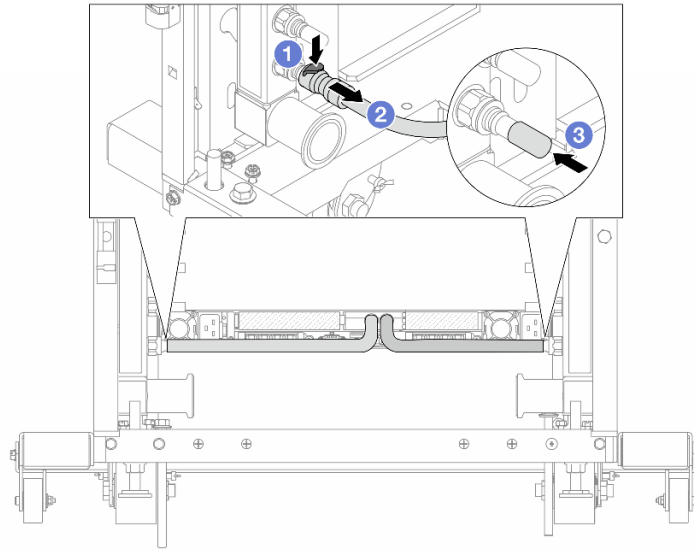
Figura 163. Extracción de los conectores rápidos
