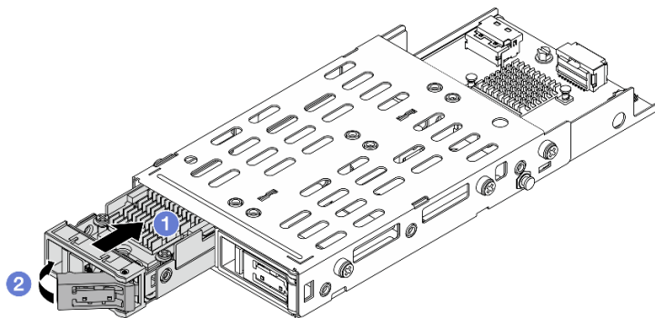
Figura 215. Instalación del conjunto de la unidad M.2
