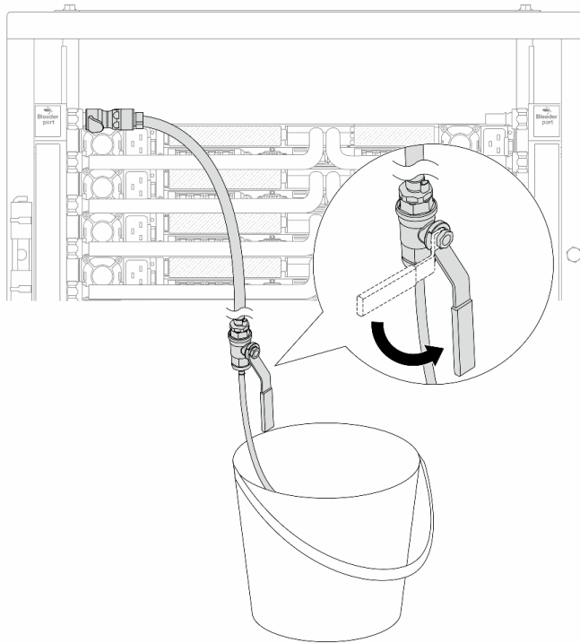
Figura 158. Apertura de la válvula de purga del lado de suministro
