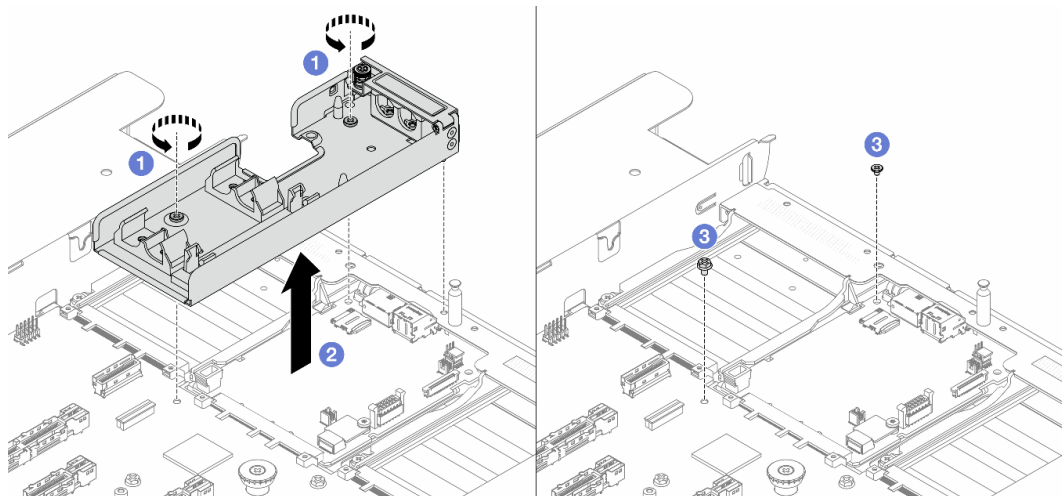
Figura 122. Extracción del soporte
