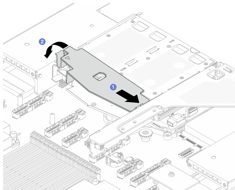
Figura 63. Instalación del deflector de aire
