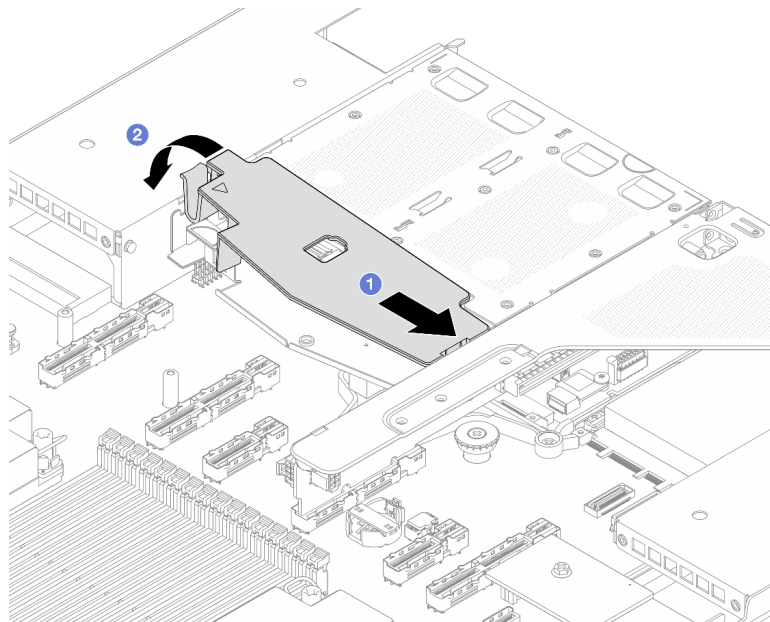
Figura 204. Instalación del deflector de aire
