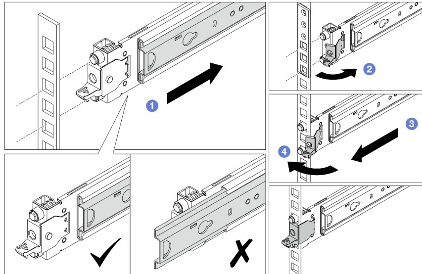
Figura 32. Instalación de las patillas de montaje frontales
