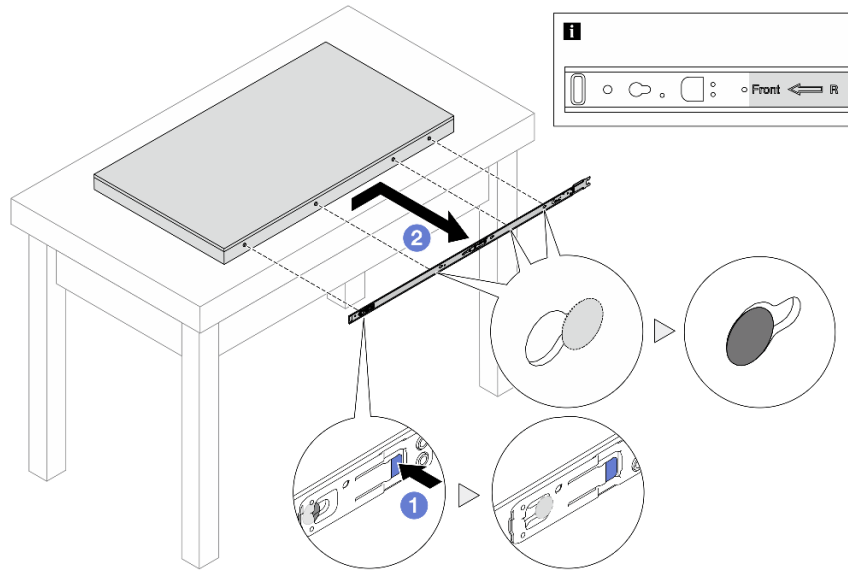
Figura 48. Extracción de los rieles internos
