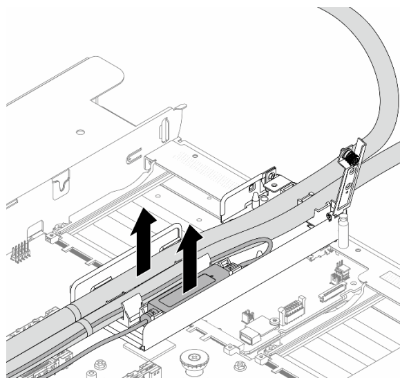
Figura 120. Desenganche de las mangueras y el módulo
