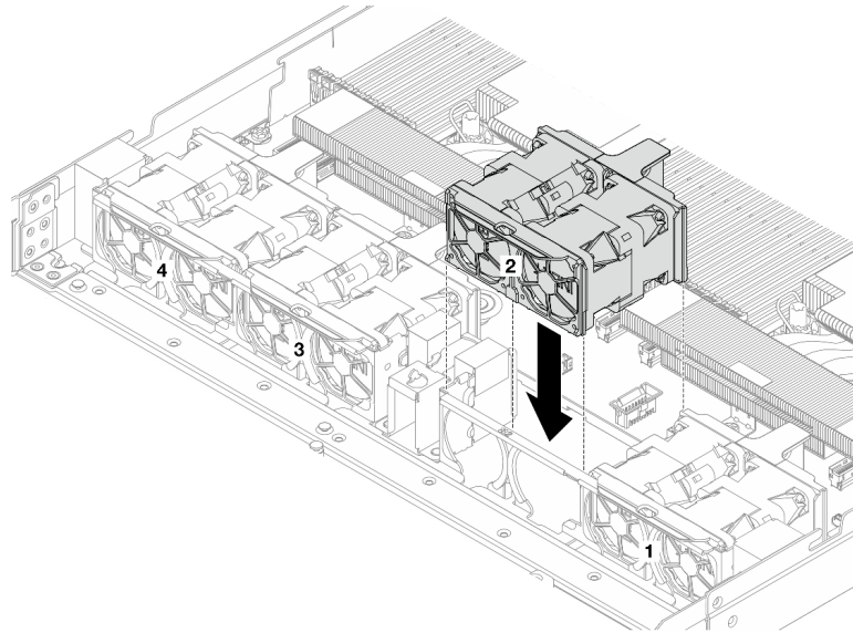
Figura 114. Reinstalación del paquete de ventiladores 2
