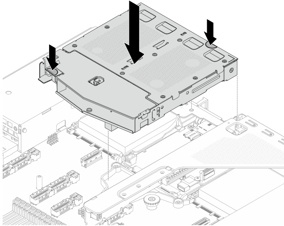
Figura 205. Instalación del compartimiento de la unidad trasera de 2,5"
