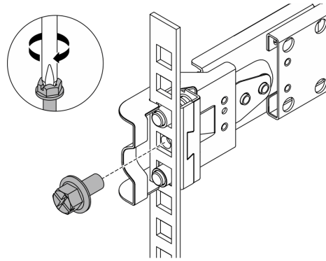
Figura 55. Fijación del servidor en la parte posterior del bastidor
