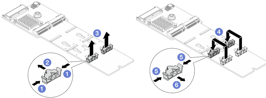
Figura 104. Ajuste del elemento de sujeción M.2
