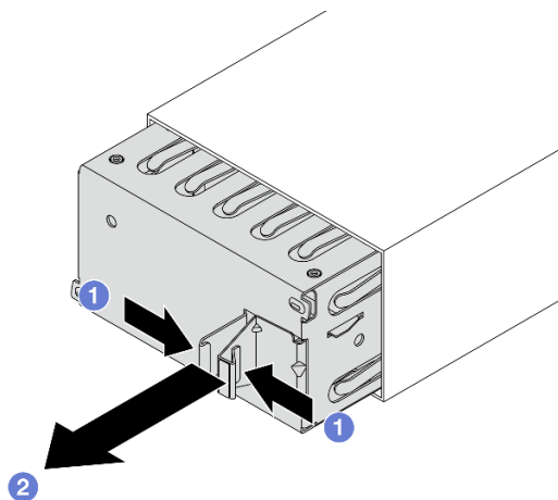
Figura 99. Extracción de relleno de la unidad de fuente de alimentación de intercambio en caliente
