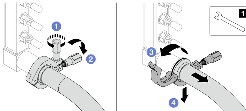
Figura 169. Separación del múltiple del kit de manguera
