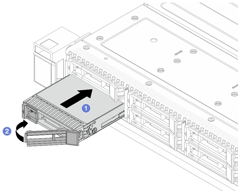
Figura 94. Instalación de unidad de intercambio en caliente
