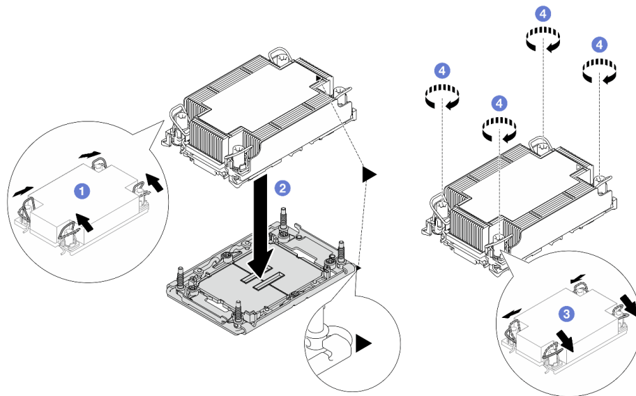
Figura 197. Instalación de un PHM
