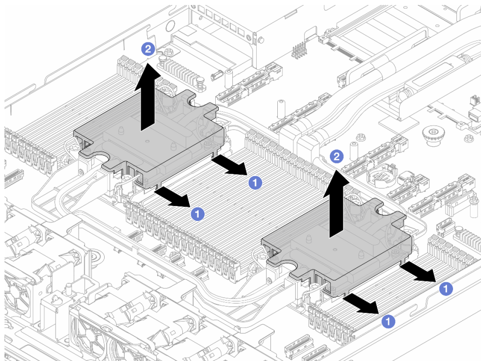
Figura 293. Extracción de la cubierta de la placa de frío
