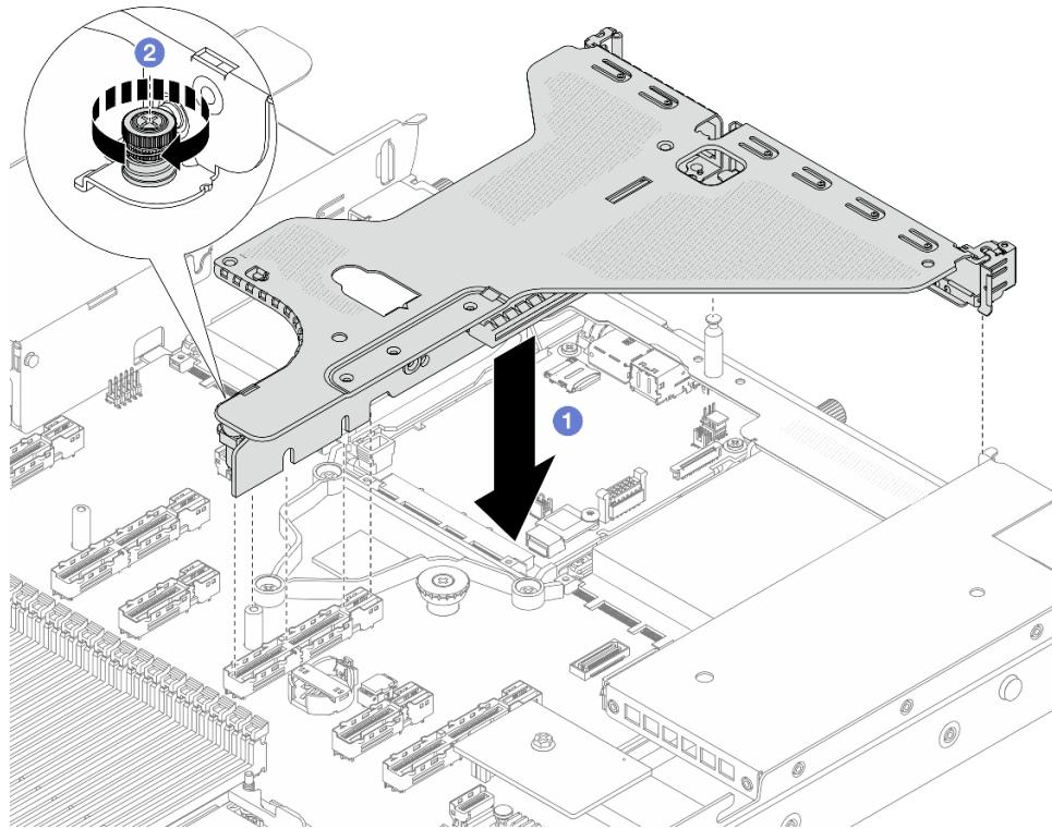
Figura 264. Instalación del conjunto de expansión
