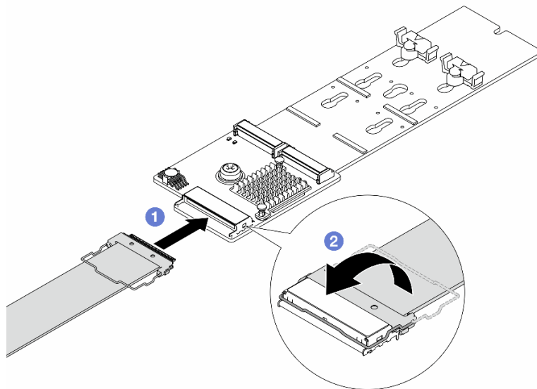
Figura 108. Conexión del cable M.2
