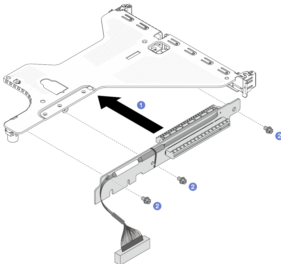
Figura 263. Instalación de la tarjeta de sujeción
