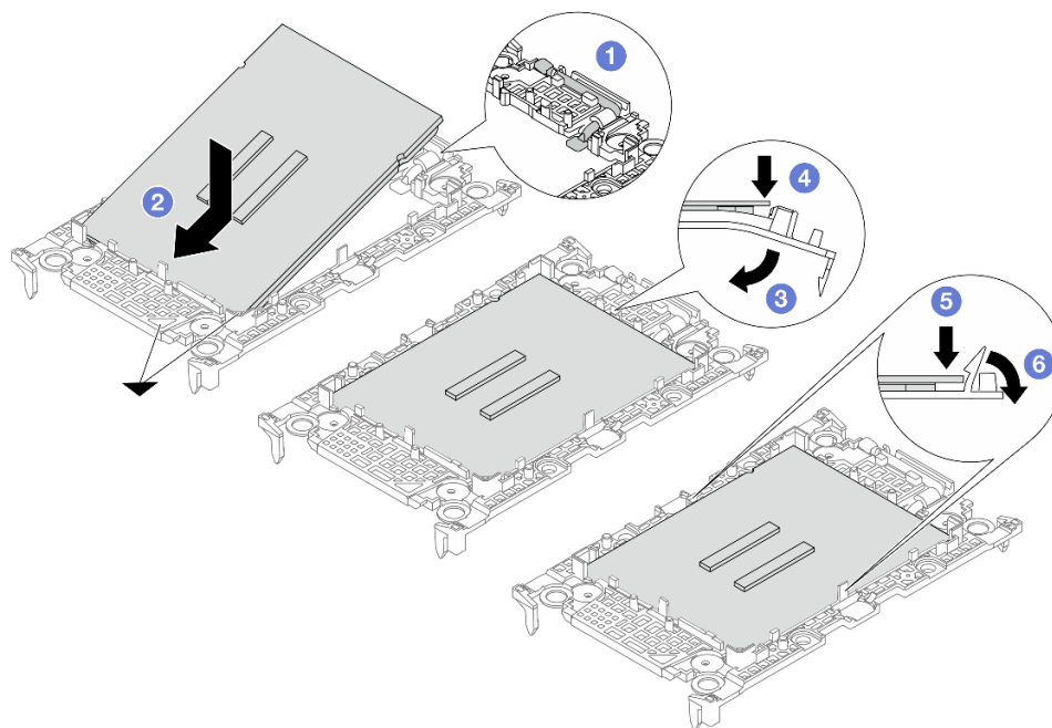
Figura 193. Instalación de un transportador de procesador
