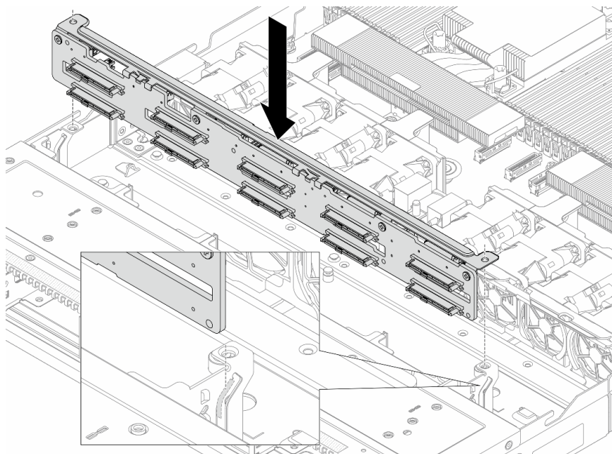
Figura 59. Instalación de la placa posterior de diez unidades de intercambio en caliente de 2,5”
