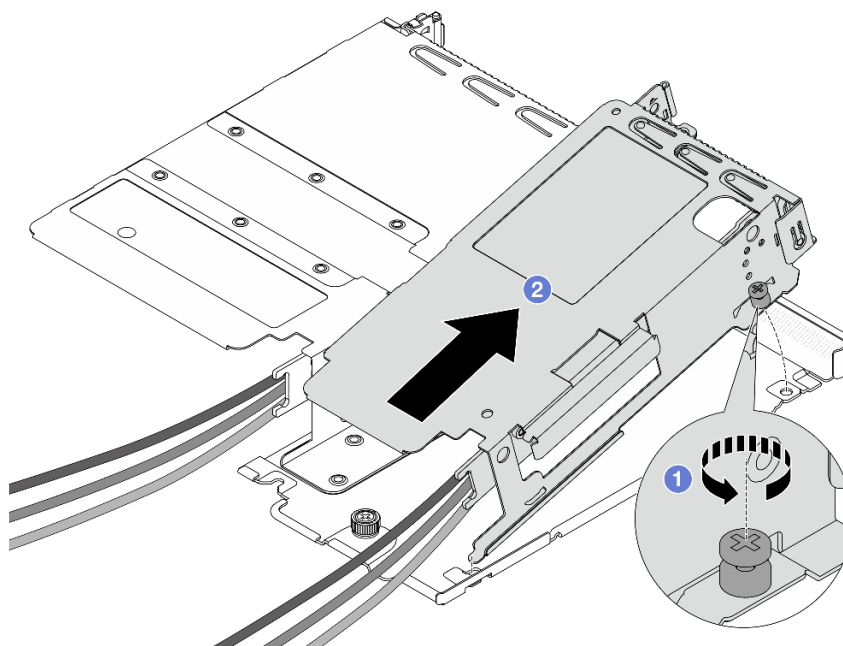
Figura 73. Separación de los dos compartimientos
