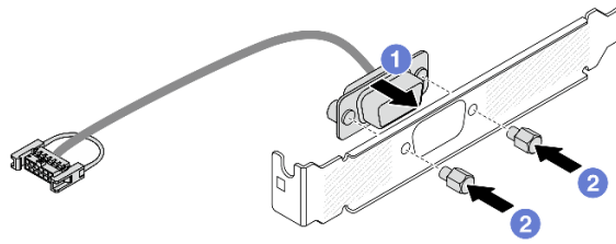
Figura 273. Ensamblaje del módulo de puerto serie
