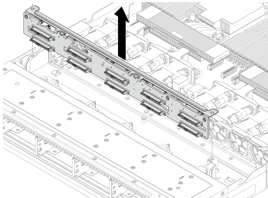
Figura 58. Extracción de la placa posterior de diez unidades de 2,5” de intercambio en caliente
