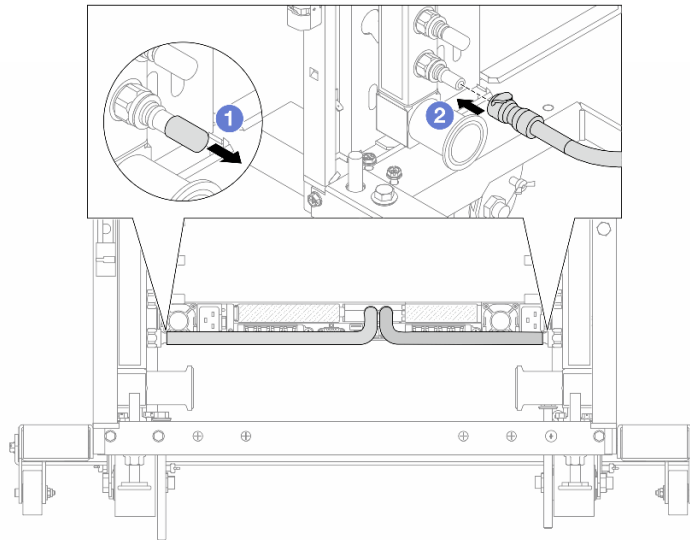
Figura 171. Instalación del conector rápido
