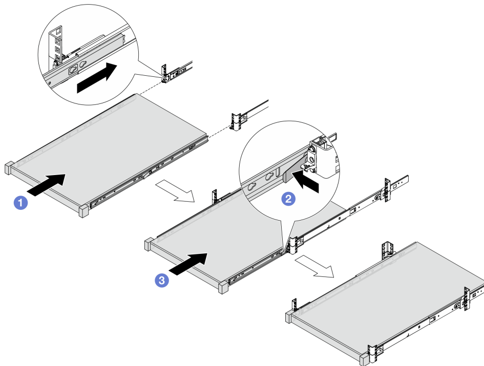
Figura 42. Instalación del servidor
