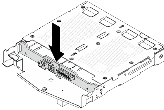
Figura 203. Instalación de la placa posterior
