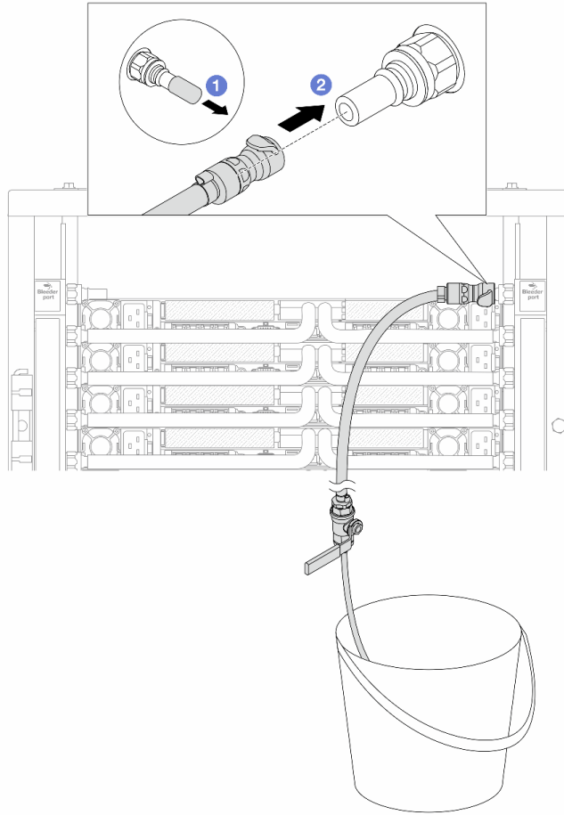
Figura 176. Instalación del kit de purga en el lado de retorno
