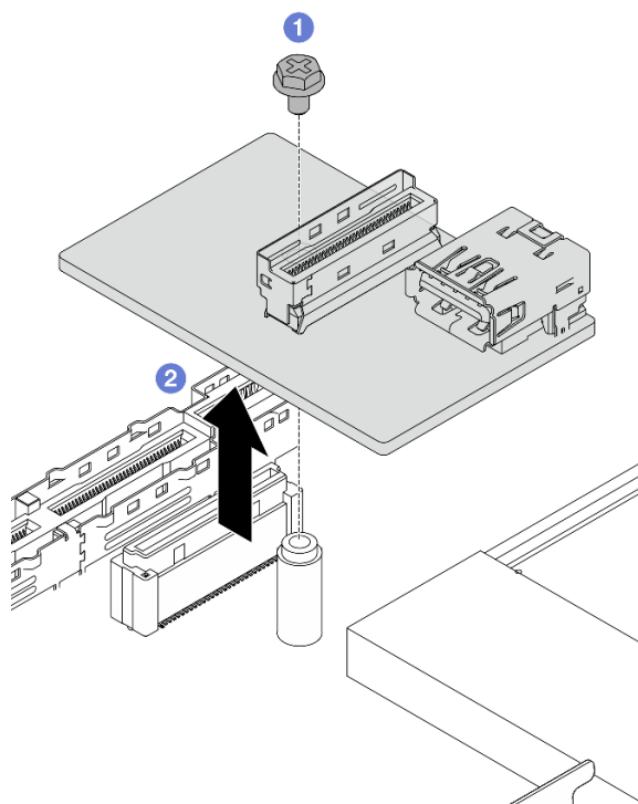
Figura 287. Extracción de la placa de E/S USB
