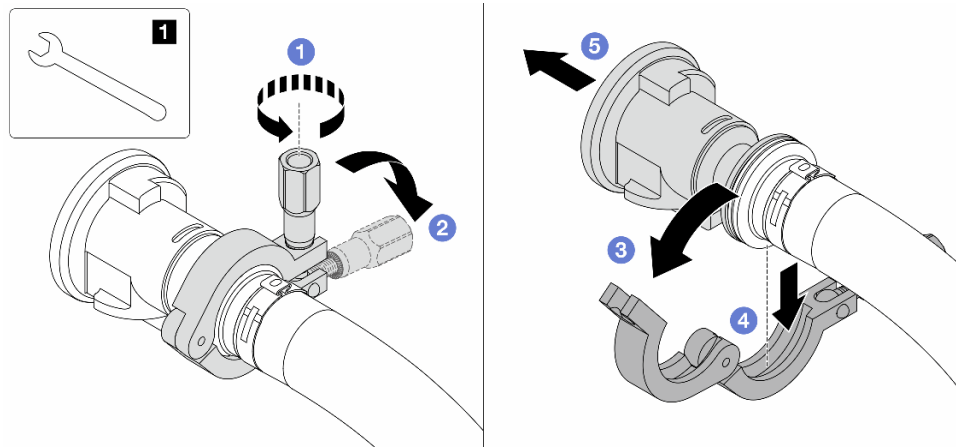
Figura 149. Separación de válvulas de bola
