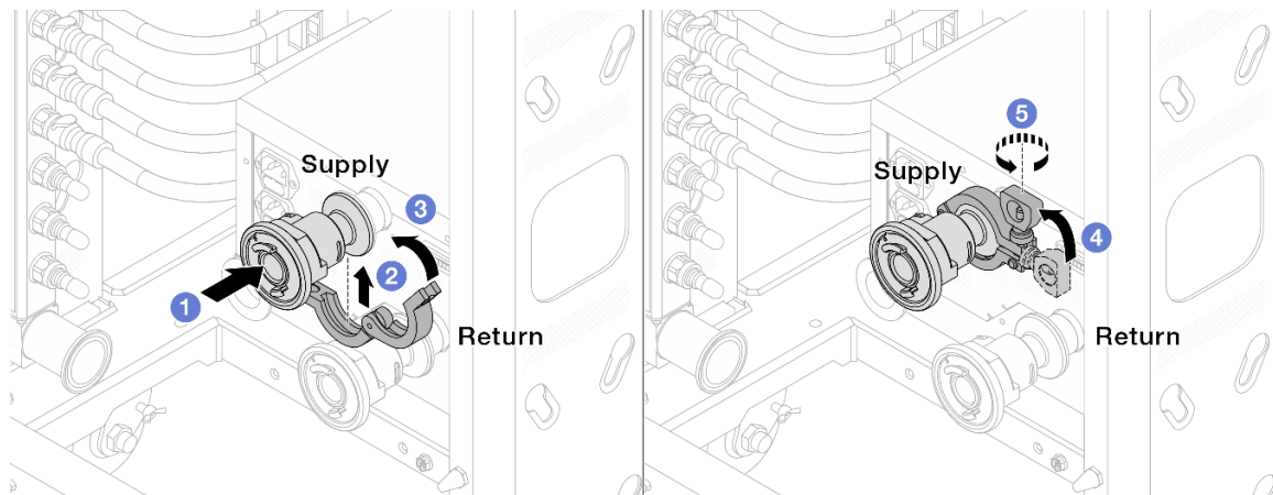
Figura 150. Instalación de válvulas de bola
