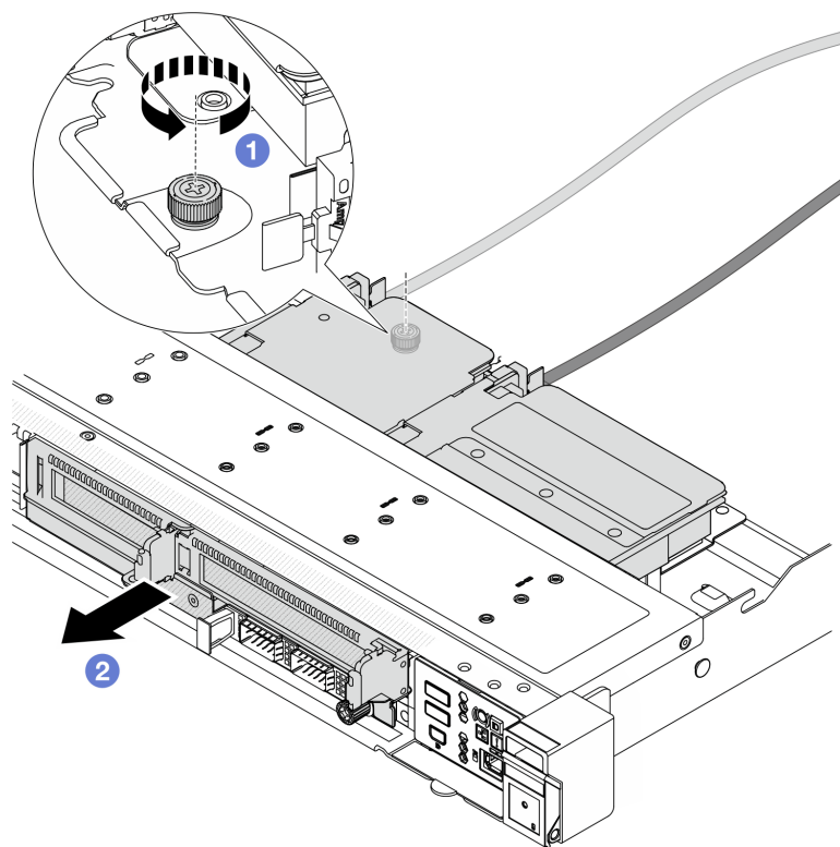
Figura 71. Extracción del compartimiento de expansión frontal
