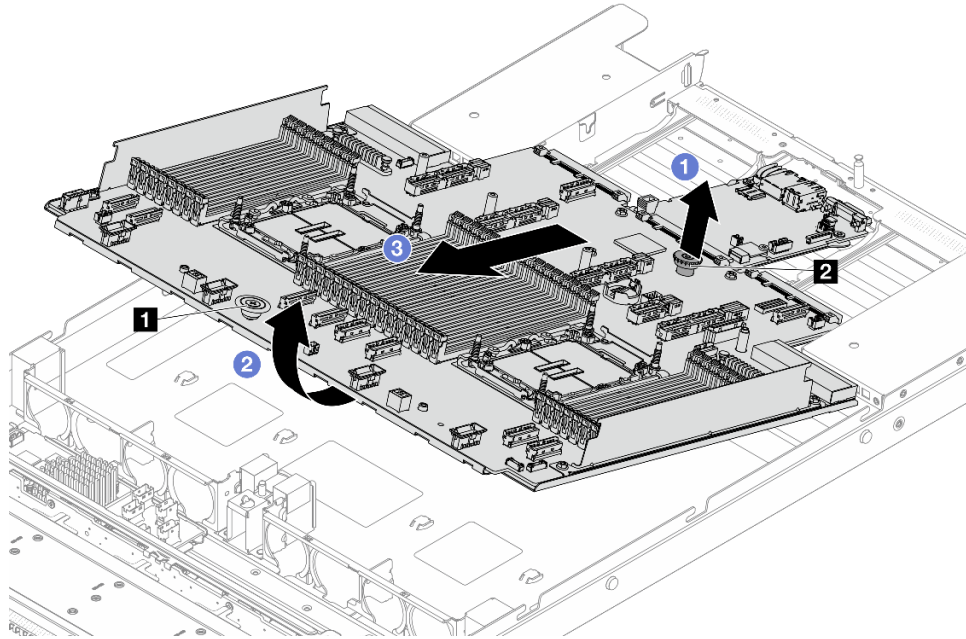
그림 281. 시스템 보드 어셈블리 제거
