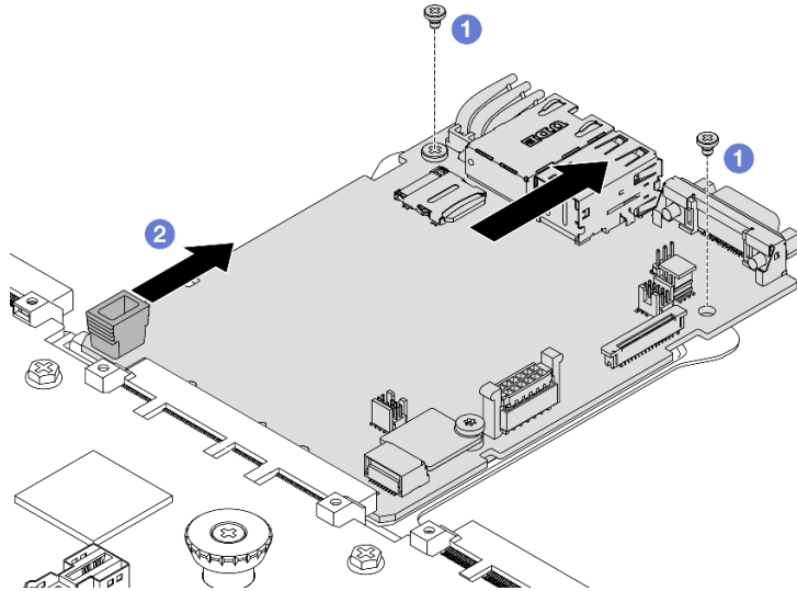
그림 279. 시스템 I/O 보드 제거
