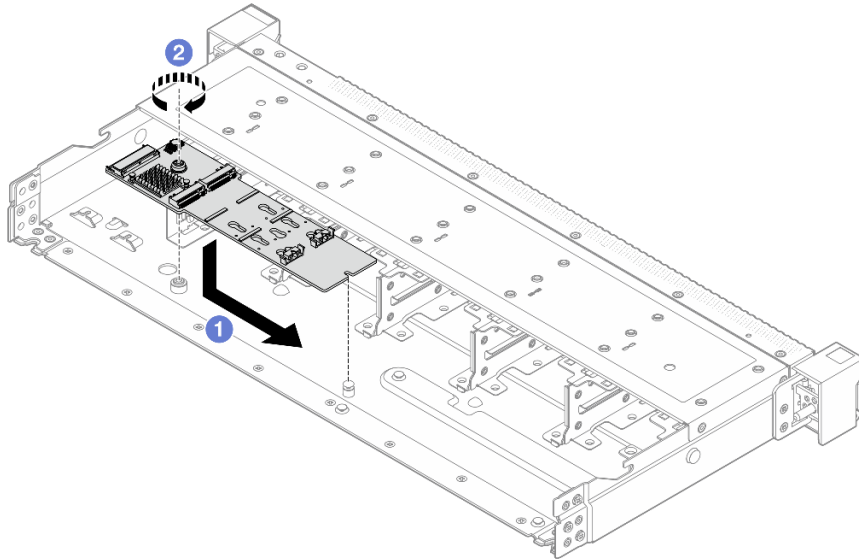
그림 108. M.2 백플레인 설치
