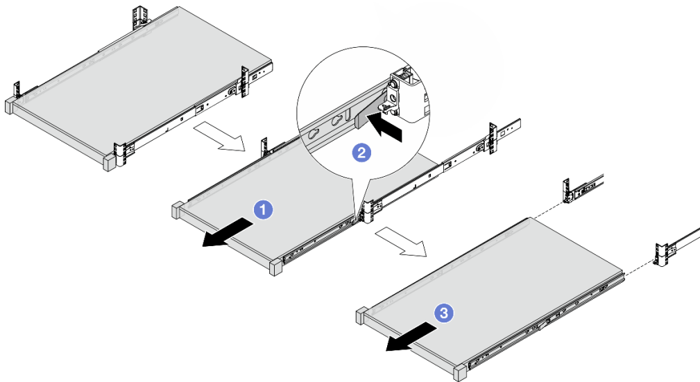
그림 37. 서버 제거
