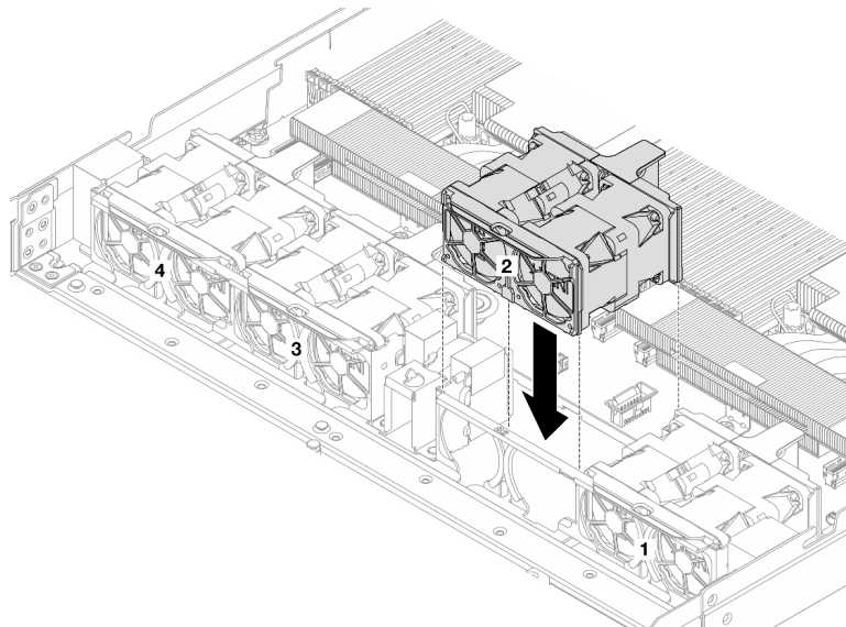
그림 113. 팬 팩 2 재설치
