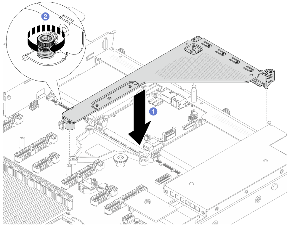
그림 277. 라이저 어셈블리 설치
