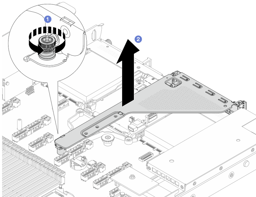
그림 272. 라이저 브래킷 제거
