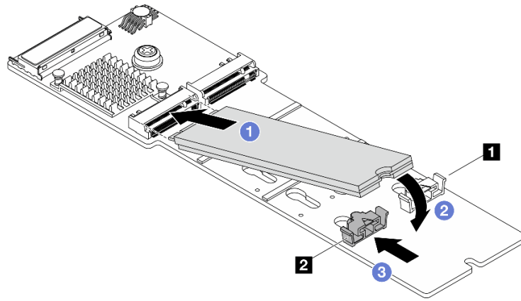
그림 109. M.2 드라이브 설치
