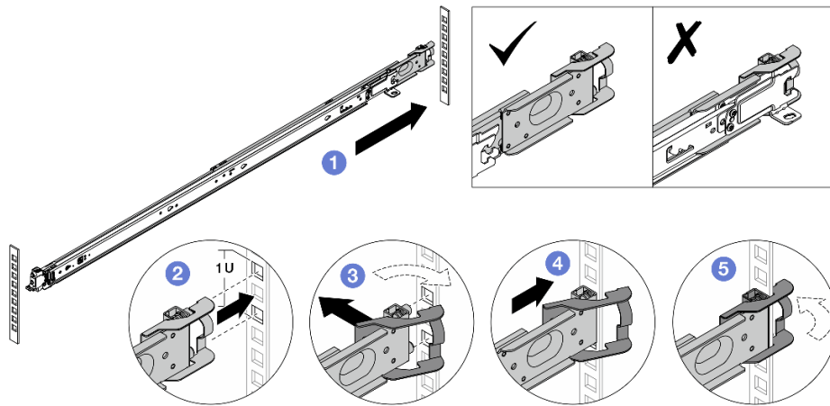
그림 33. 뒷면 마운팅 핀 설치
