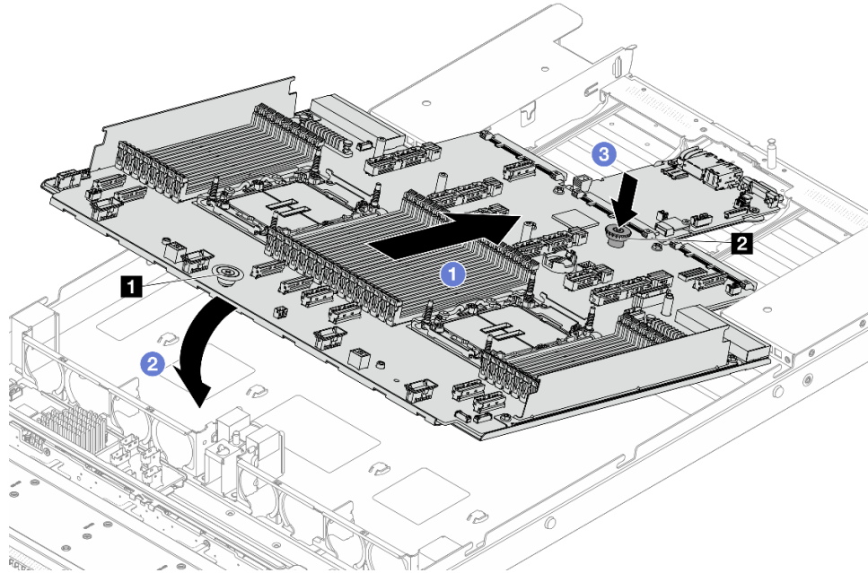
그림 283. 시스템 보드 어셈블리 설치
