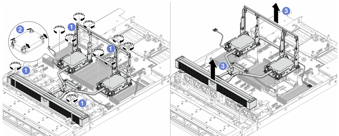
그림 118. NeptAir 모듈 제거
