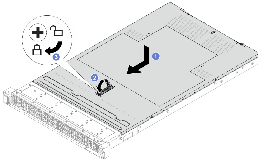
그림 287. 윗면 덮개 설치
