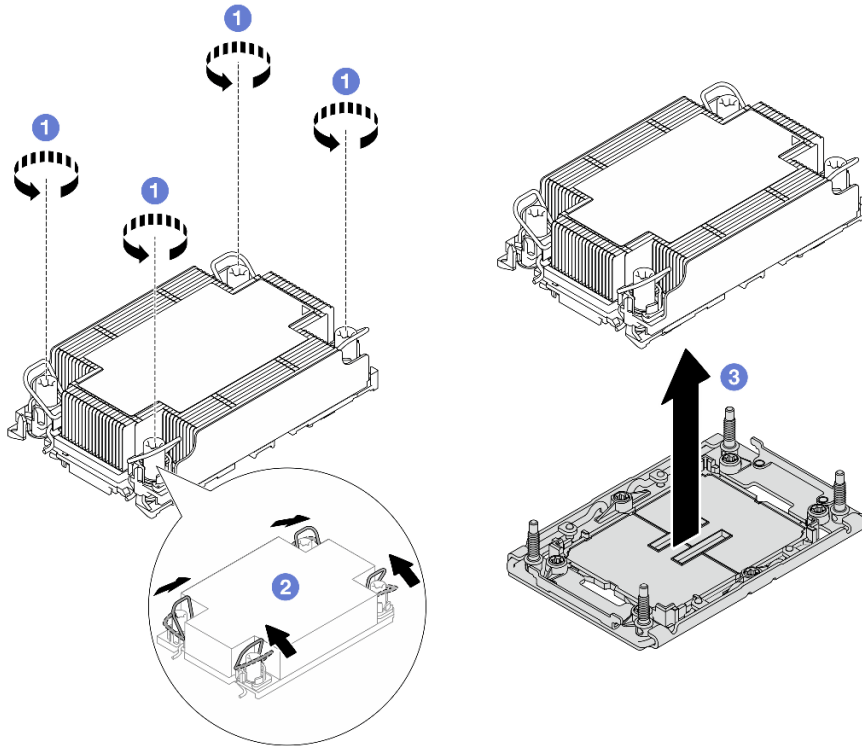
그림 192. PHM 제거
