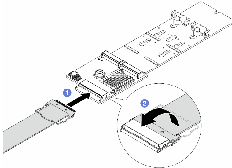
그림 110. M.2 케이블 연결
