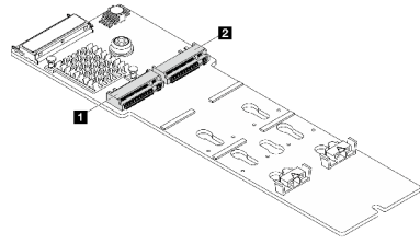
그림 107. M.2 드라이브 슬롯
