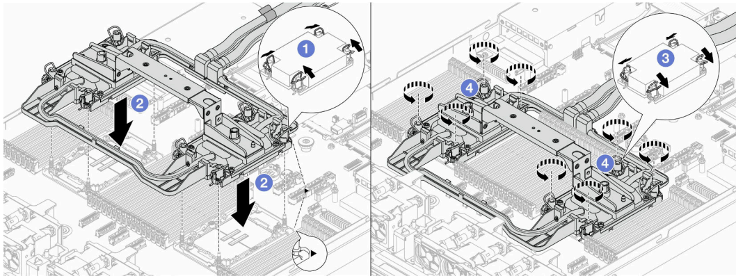
그림 130. NeptCore 모듈 설치
