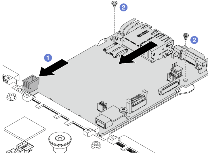
그림 280. 시스템 I/O 보드 설치
