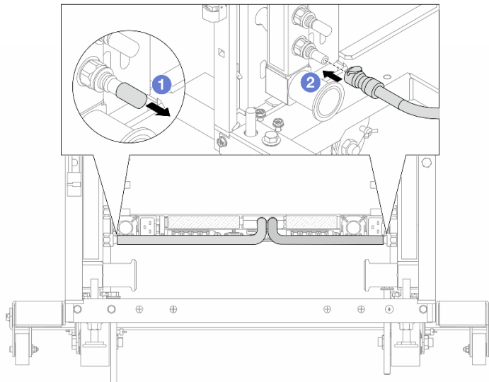
그림 158. 퀵 커넥트 플러그 설치
