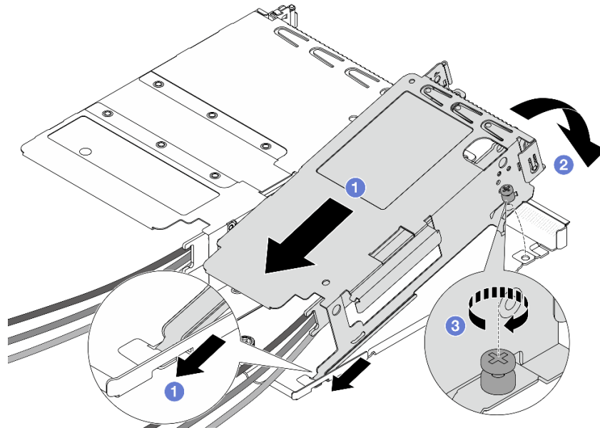
그림 80. 두 라이저 케이스 조립
