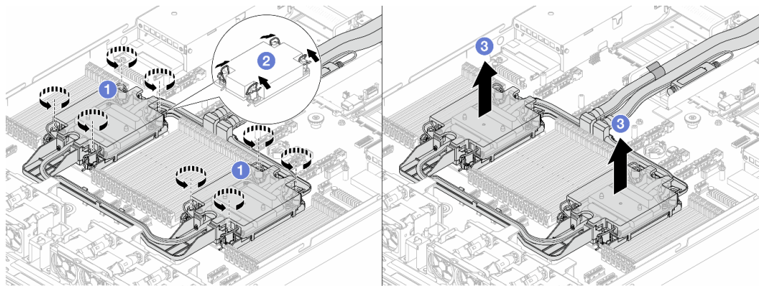
그림 124. NeptCore 모듈 제거
