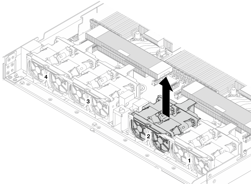
그림 284. 시스템 팬 팩 제거
