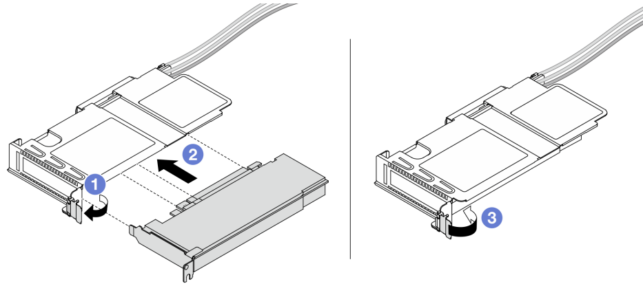
그림 79. PCIe 어댑터 설치
