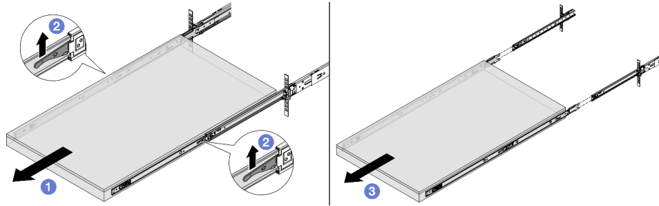
그림 47. 서버 꺼내기
