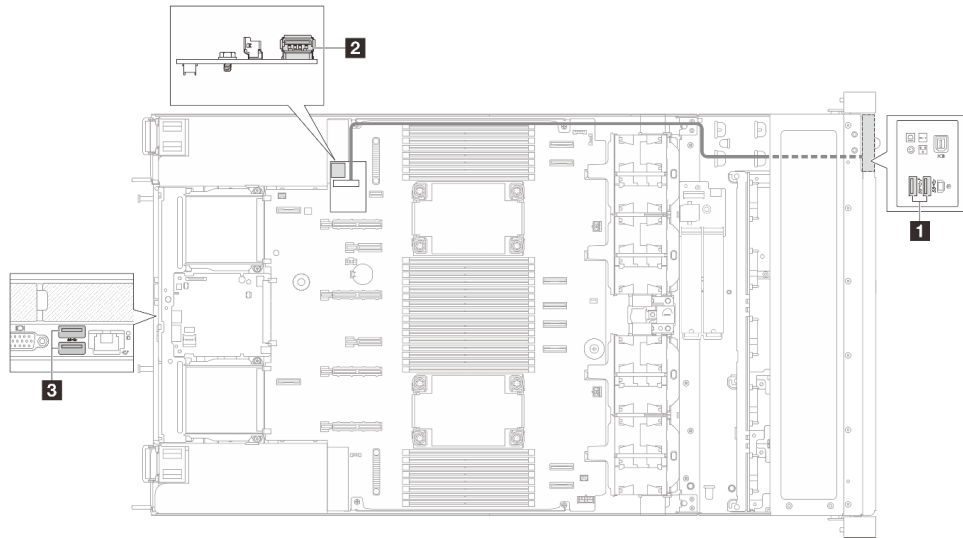
그림 307. USB 포트 개요
