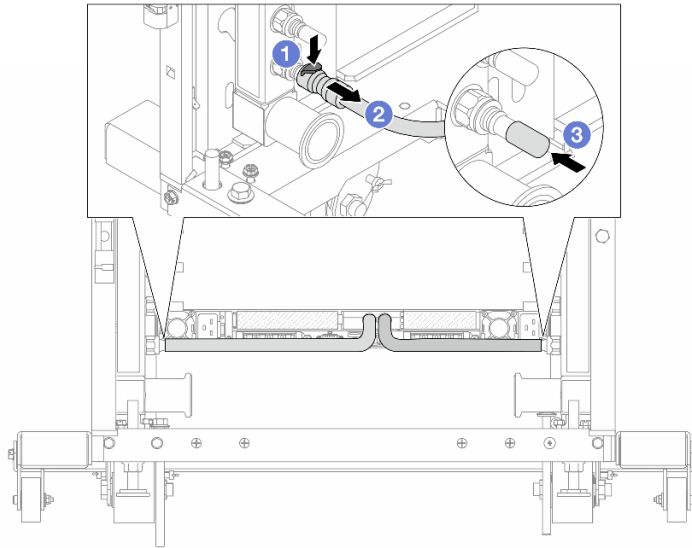
그림 143. 퀵 커넥트 플러그 제거
