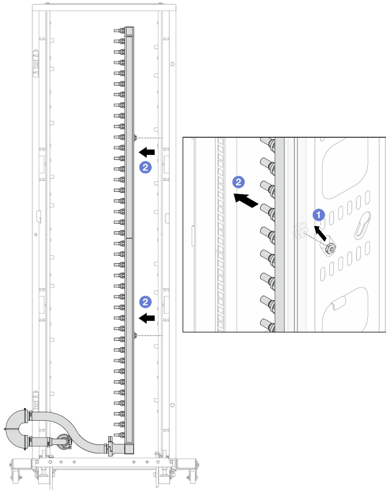
그림 145. 매니폴드 제거
