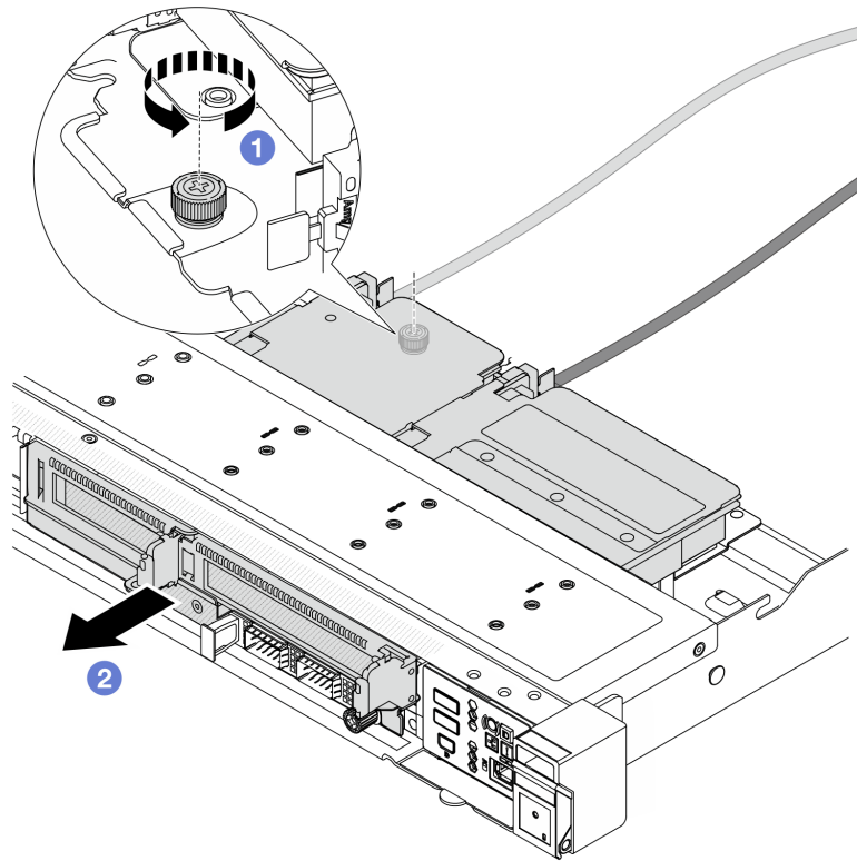
그림 71. 앞면 라이저 케이스 제거
