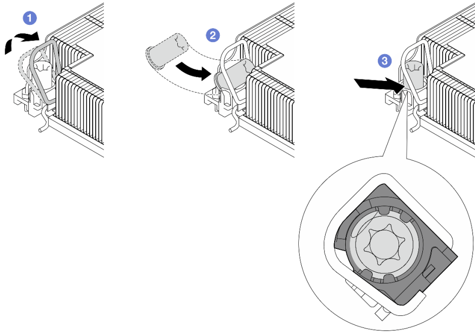
그림 90. 방열판에 Torx T30 너트 설치
