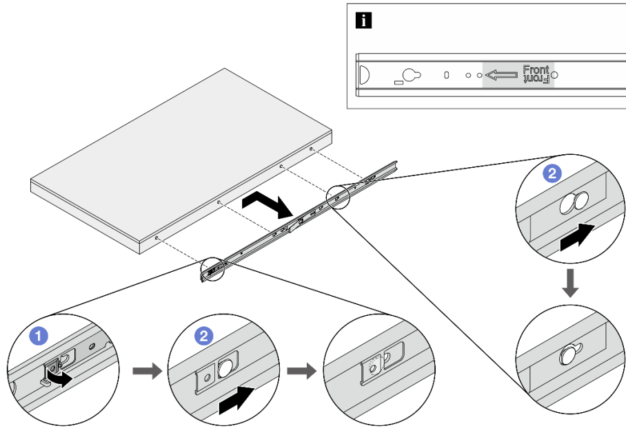
그림 38. 내부 레일 제거
