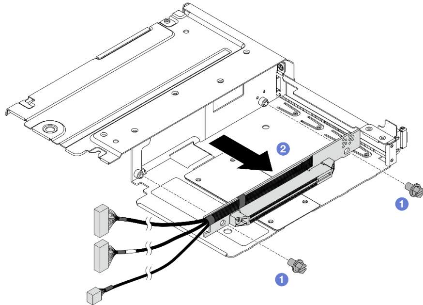
그림 76. 전체 높이 케이스에서 라이저 카드 제거
