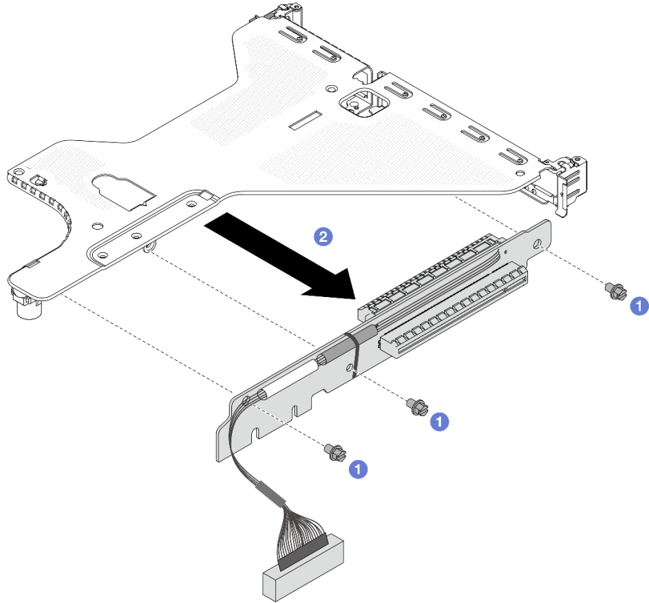
그림 264. 라이저 카드 제거
