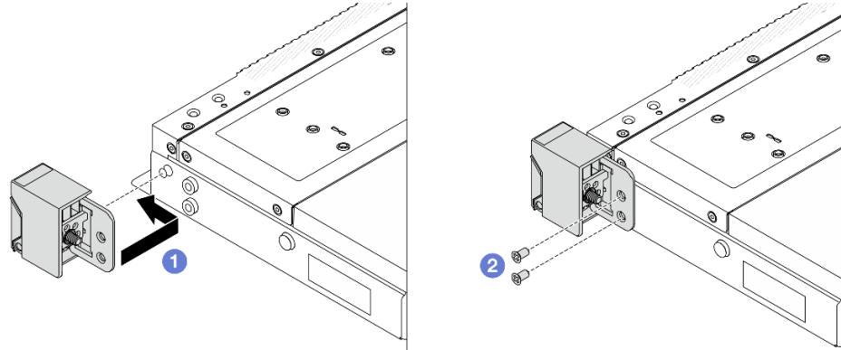
그림 203. 랙 래치 설치
