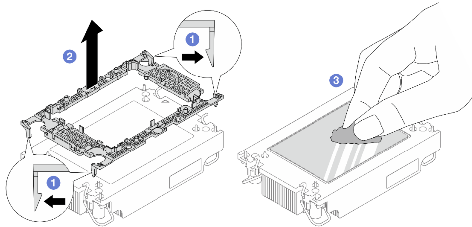
그림 194. 방열판에서 프로세서 캐리어 분리 중
