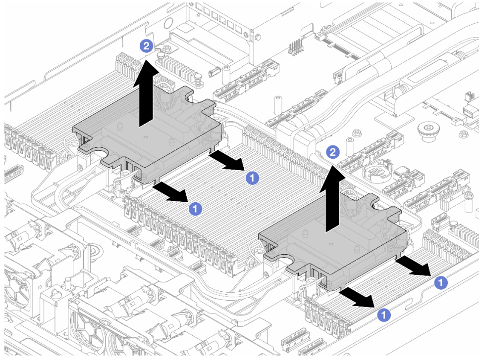
그림 306. 냉각팬 덮개 제거
