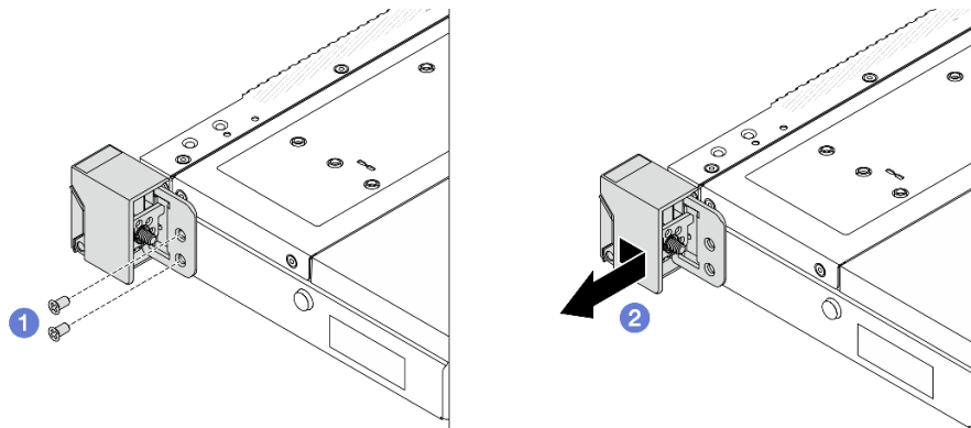
그림 202. 랙 래치 제거
