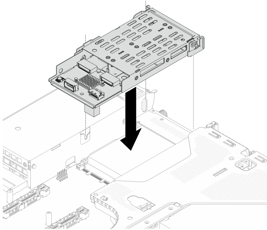
그림 223. M.2 케이스 설치
