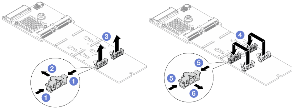
그림 106. M.2 고정장치 조정
