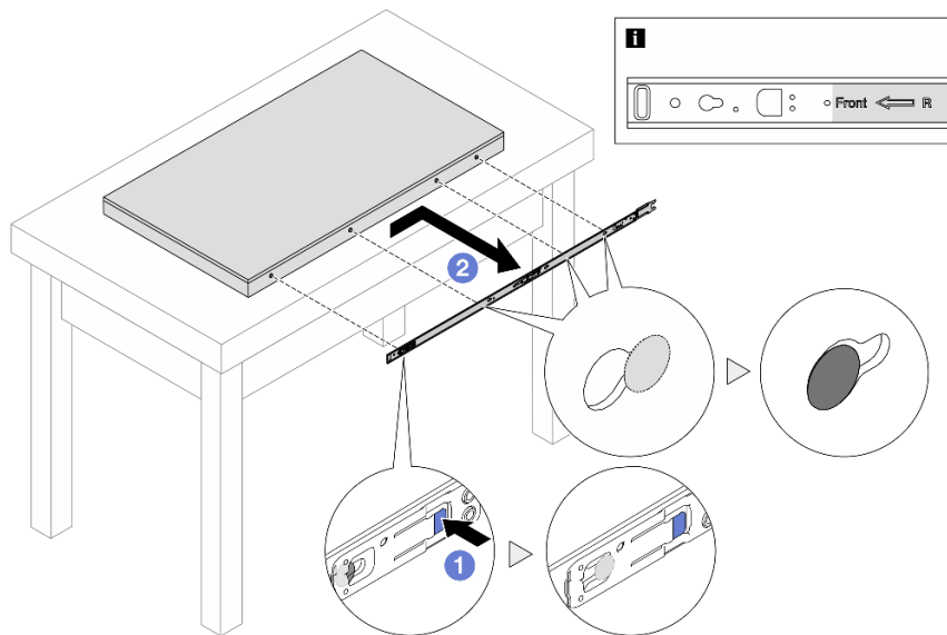
그림 48. 내부 레일 제거
