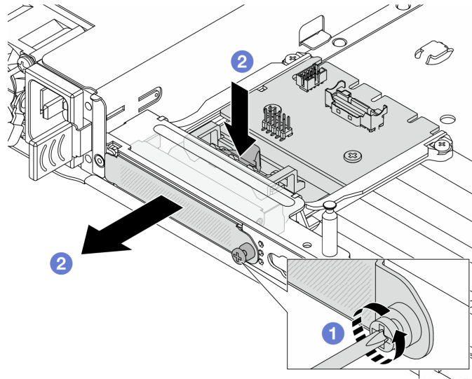
그림 85. 뒷면 OCP 인터포저 카드 제거
