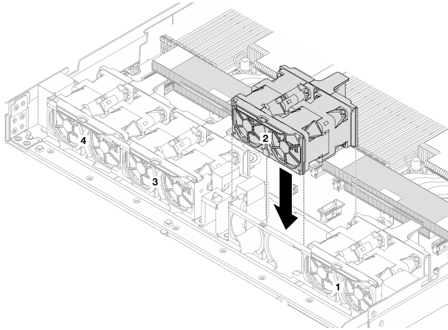
그림 285. 시스템 팬 팩 설치
