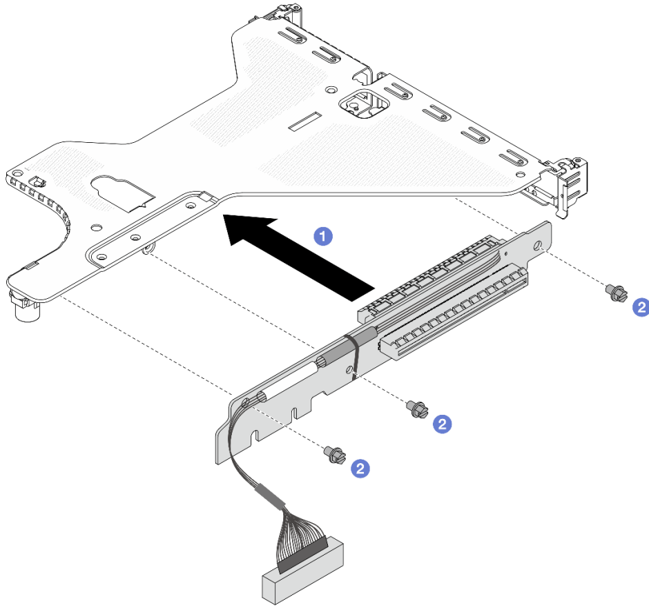
그림 265. 라이저 카드 설치
