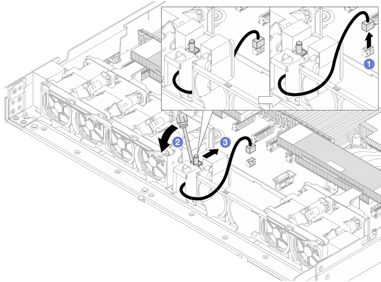
그림 112. 침입 스위치 제거
