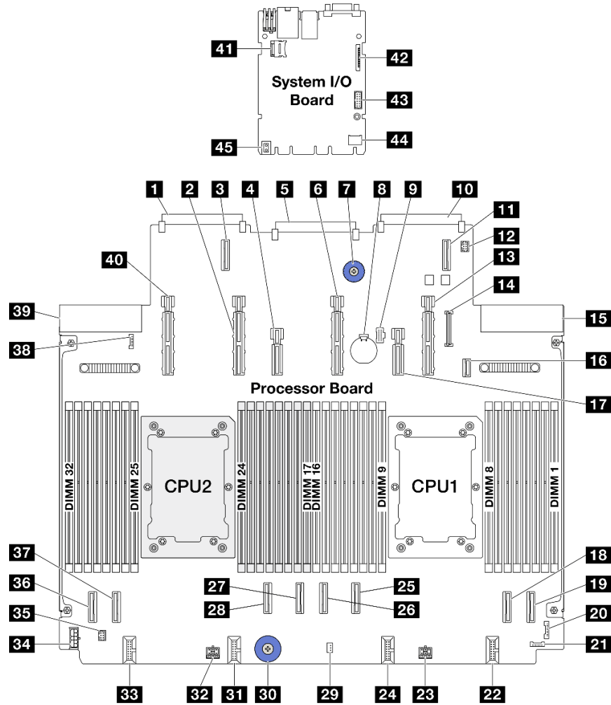
그림 292. 시스템 보드 어셈블리 커넥터
