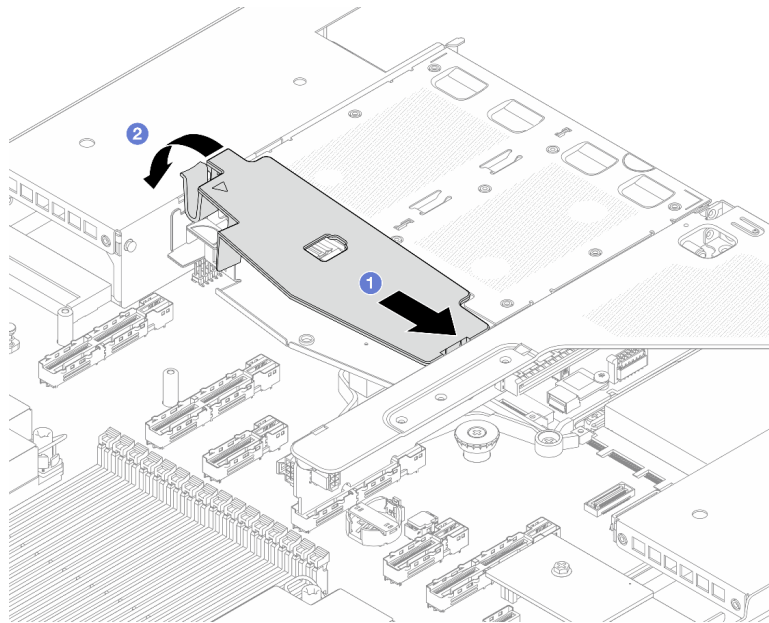
그림 63. 공기 조절 장치 설치
