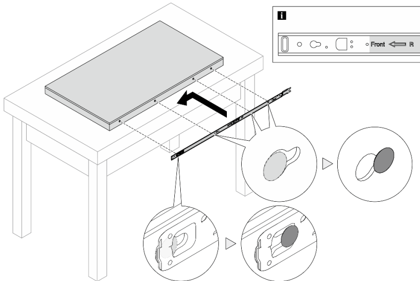
그림 50. 내부 레일 설치
