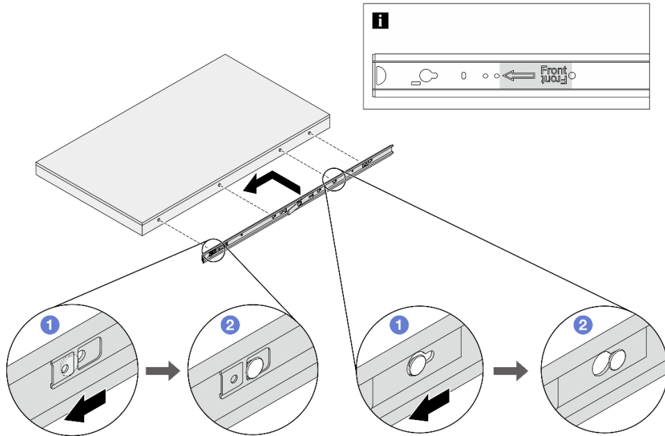
그림 40. 내부 레일 설치
