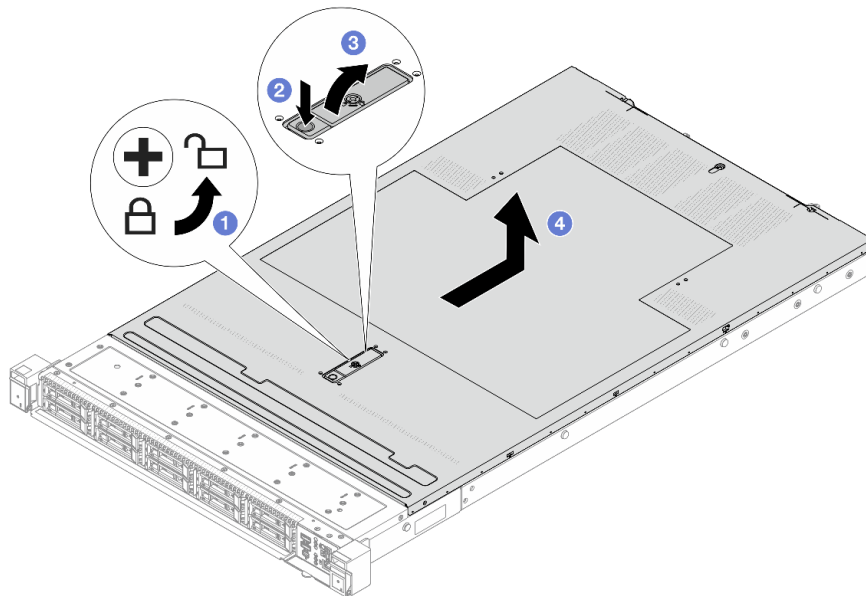
그림 286. 윗면 덮개 제거
