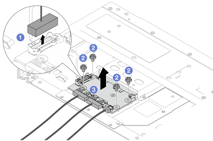
그림 83. 앞면 OCP 인터포저 카드 제거
