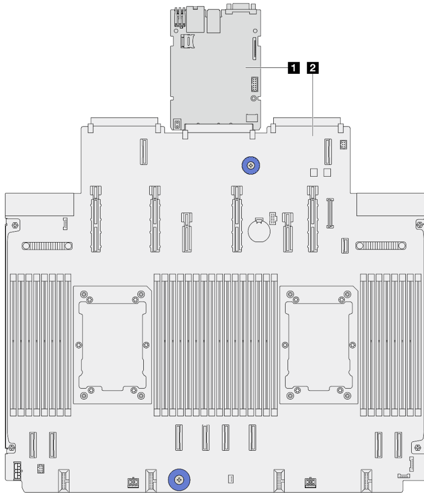
그림 278. 시스템 보드 어셈블리 레이아웃
