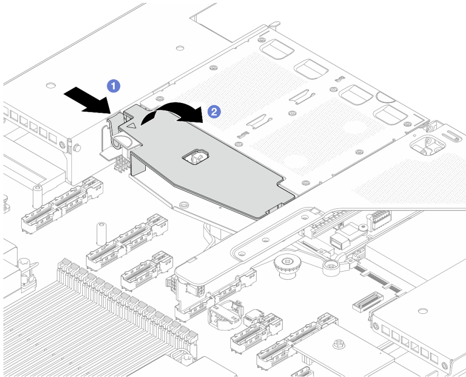
Рис. 60. Снятие дефлектора
