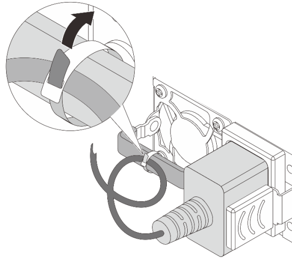
Рис. 102. Прокладка и привязывание шнура питания
