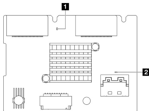
Рис. 303. Светодиодные индикаторы задней объединительной панели M.2
