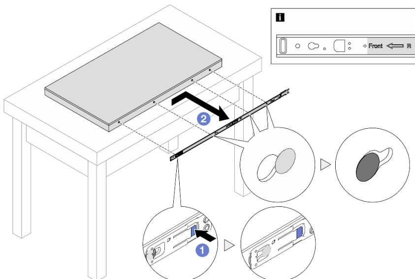
Рис. 48. Снятие внутренних направляющих
