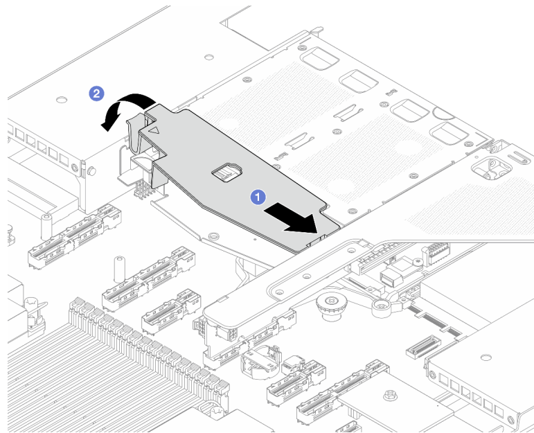
Рис. 63. Установка дефлектора
