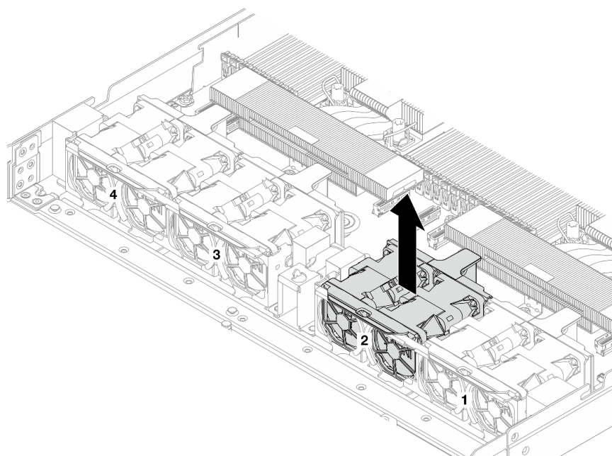
Рис. 284. Снятие блока вентиляторов компьютера
