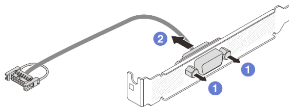
Рис. 274. Разборка модуля последовательного порта
