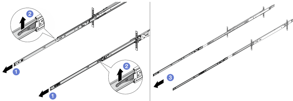
Рис. 49. Выведение направляющих
