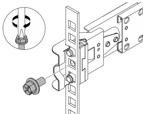
Рис. 44. Фиксация сервера на задней стороне стойки
