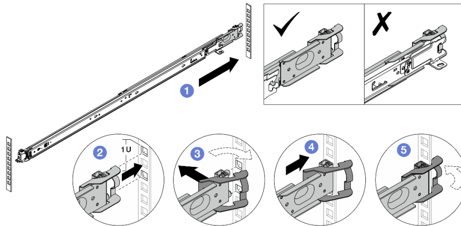
Рис. 33. Установка задних крепежных контактов
