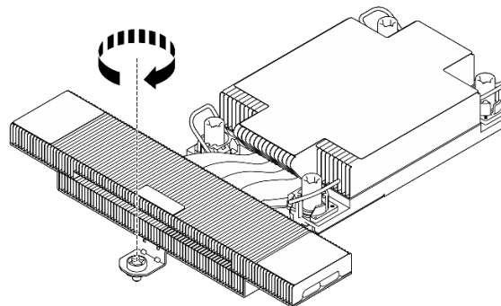
Рис. 201. Затягивание Т-образных винтов радиатора
