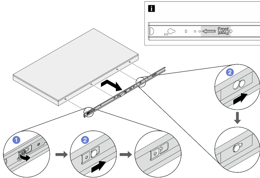
Рис. 38. Снятие внутренних направляющих
