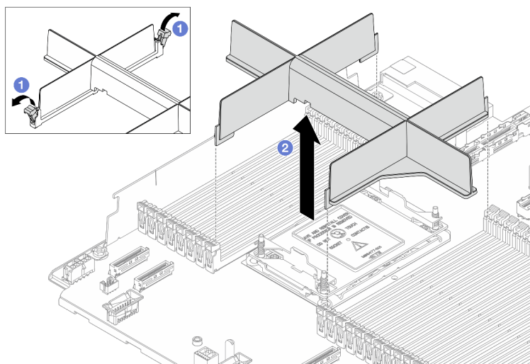
Рис. 199. Снятие заглушки PHM
