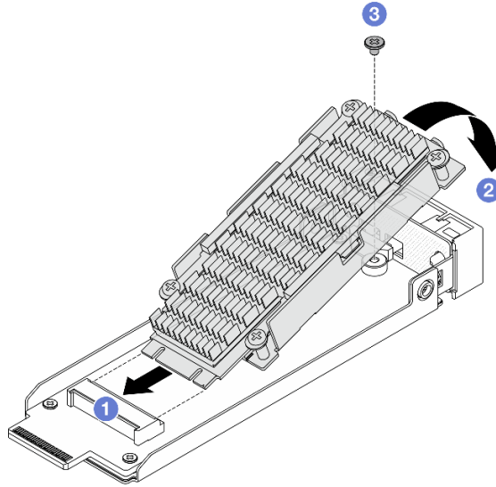
Рис. 217. Сборка интерпозера и диска M.2
