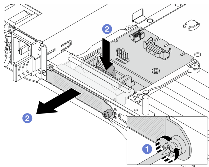
Рис. 85. Снятие задней карты интерпозера OCP
