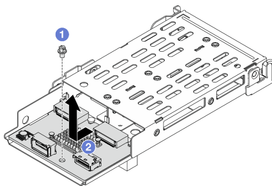
Рис. 220. Снятие объединительной панели M.2
