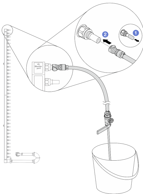
Рис. 146. Установка комплекта отводной трубки на стороне подачи
