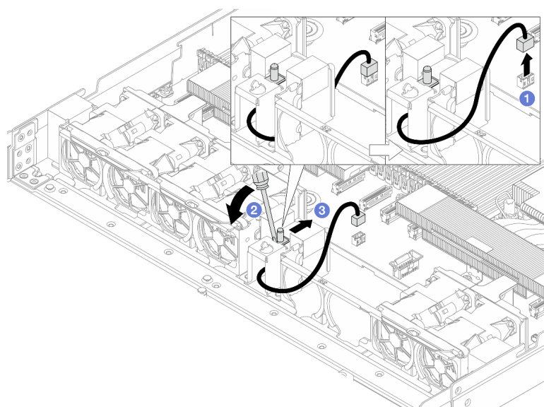
Рис. 112. Снятие датчика вмешательства
