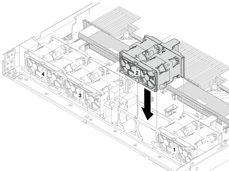
Рис. 116. Установка блока вентиляторов 2 на место
