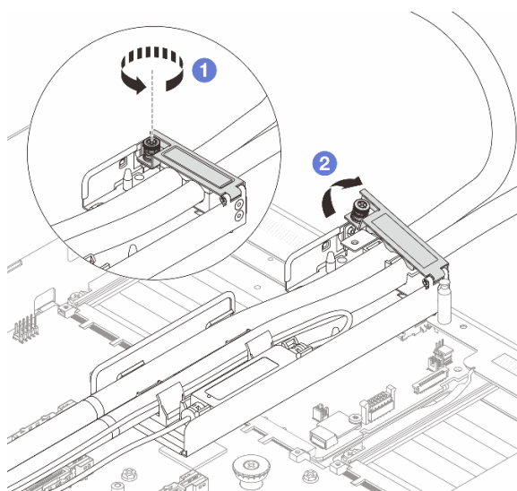
Рис. 122. Открывание кожуха держателя
