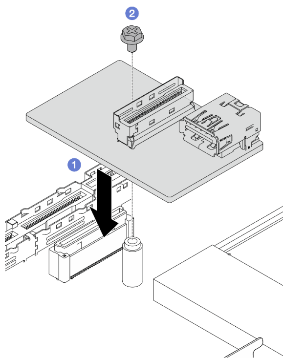
Рис. 289. Установка платы ввода-вывода USB
