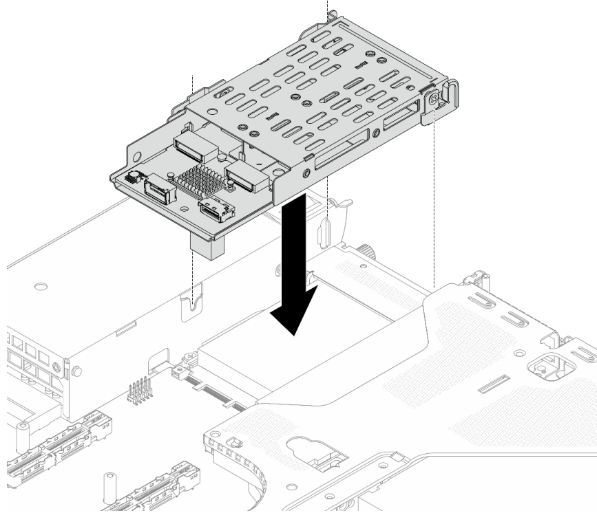
Рис. 223. Установка отсека M.2
