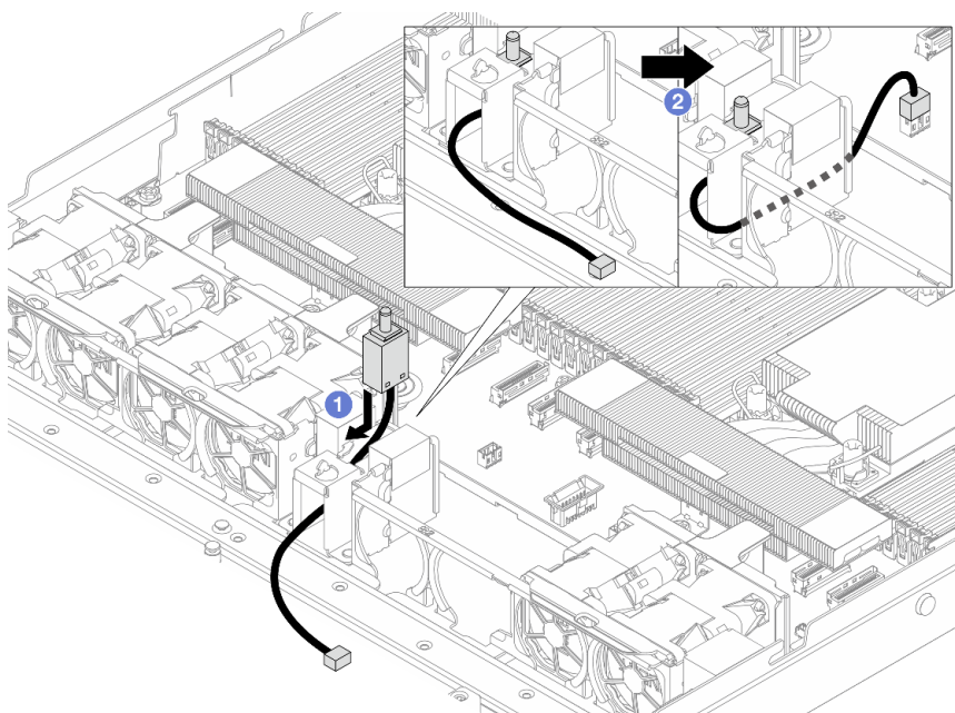
Рис. 115. Установка датчика вмешательства
