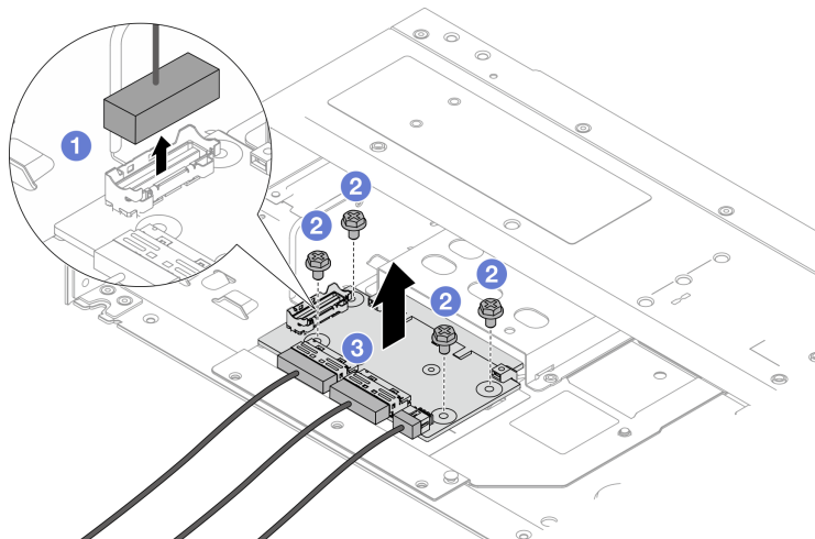
Рис. 83. Снятие передней карты интерпозера OCP
