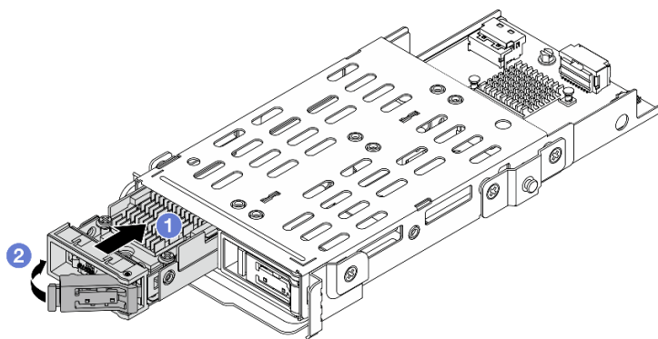
Рис. 219. Установка блока диска M.2
