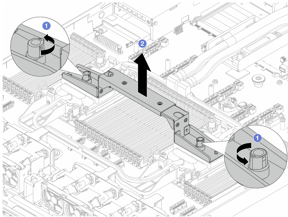
Рис. 131. Снятие ручки модуля
