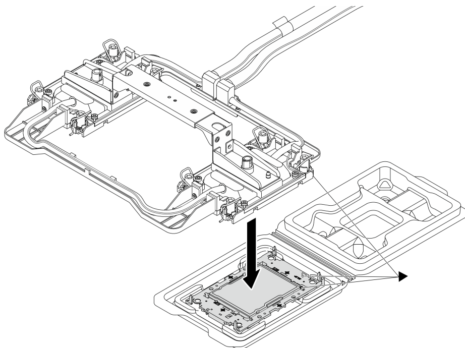
Рис. 128. Установка процессора
