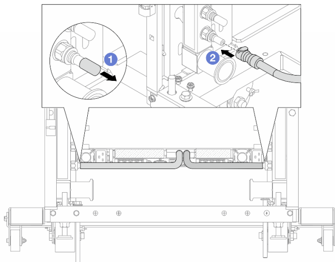
Рис. 158. Установка быстроразъемного соединителя
