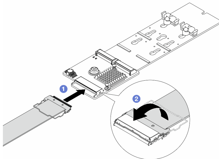
Рис. 110. Подключение кабеля M.2
