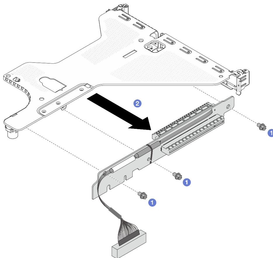
Рис. 264. Снятие платы-адаптера Riser
