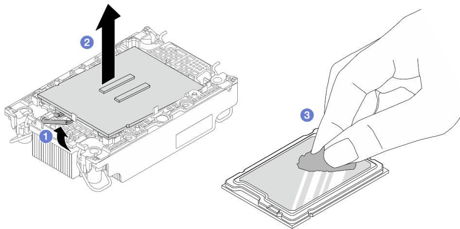
Рис. 193. Отделение процессора от радиатора и держателя
