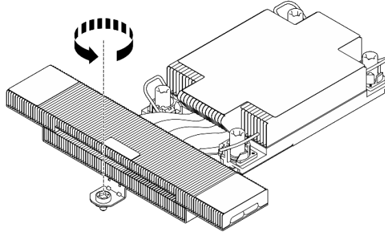
Рис. 191. Ослабление T-образных винтов радиатора
