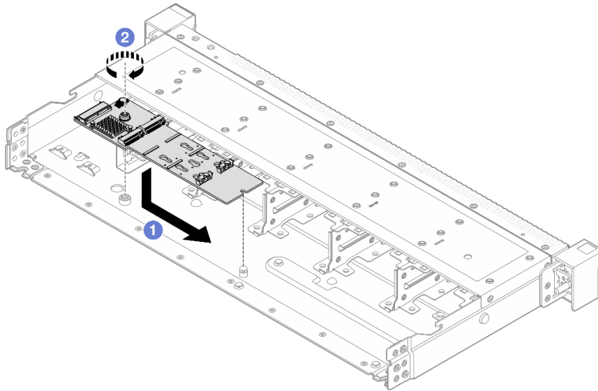
Рис. 108. Установка объединительной панели M.2
