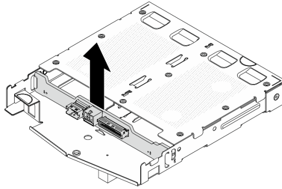
Рис. 61. Снятие задней объединительной панели для 2,5-дюймовых дисков
