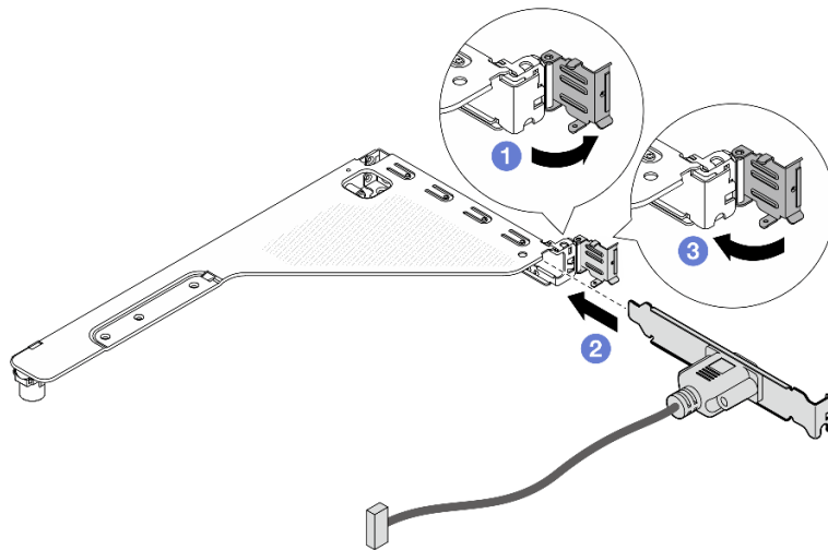
Рис. 276. Установка модуля последовательного порта
