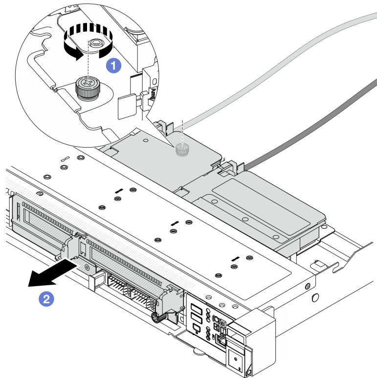
Рис. 71. Снятие переднего отсека платы-адаптера Riser
