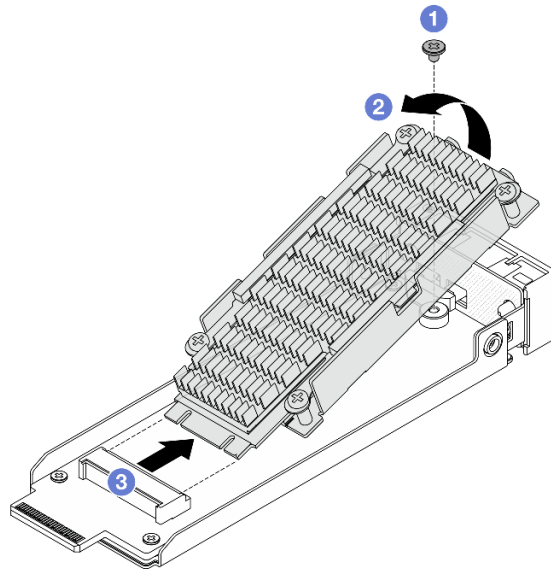
Рис. 210. Снятие интерпозера M.2 с диска
