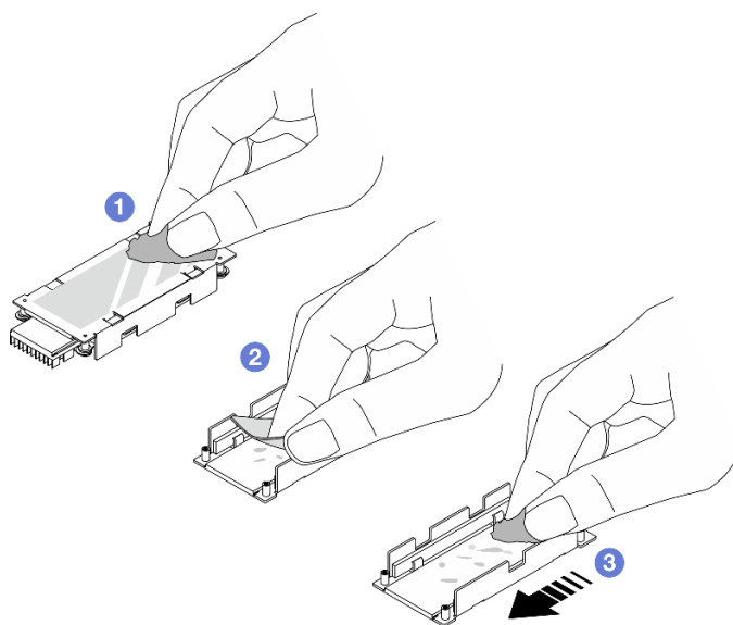
Рис. 212. Удаление термолистов
