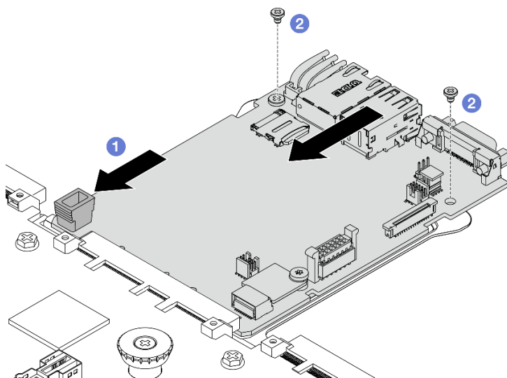
Рис. 280. Установка системной платы ввода-вывода
