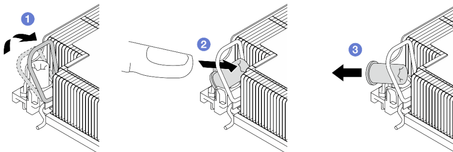
Рис. 89. Снятие гайки Torx T30 с радиатора
