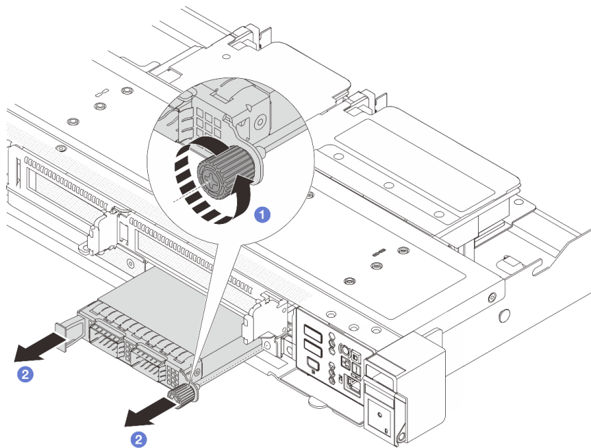
Рис. 81. Снятие переднего модуля OCP
