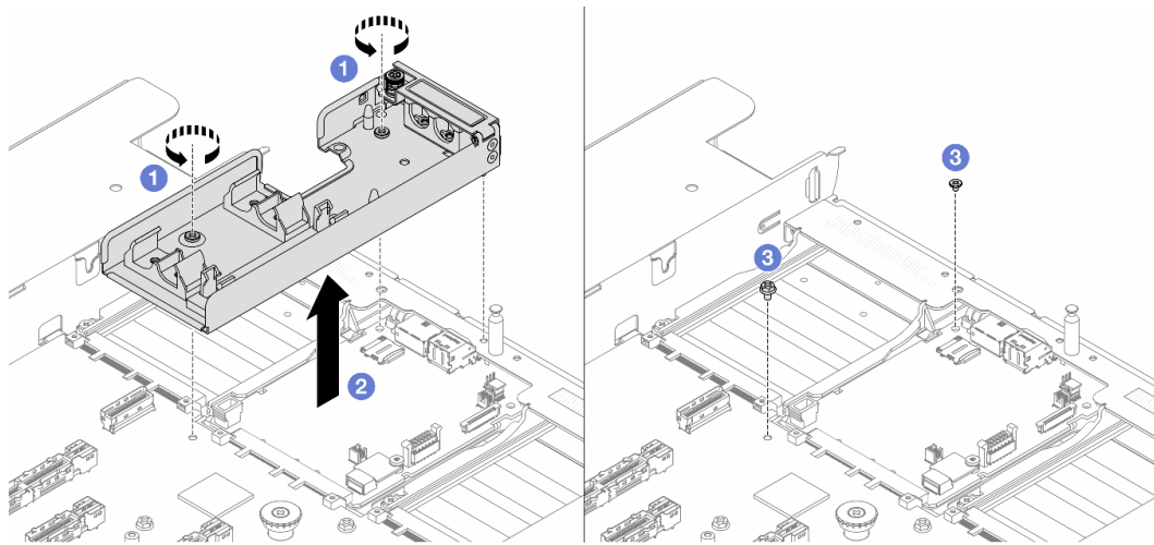
Рис. 125. Снятие держателя
