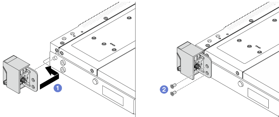
Рис. 203. Установка защелки стойки
