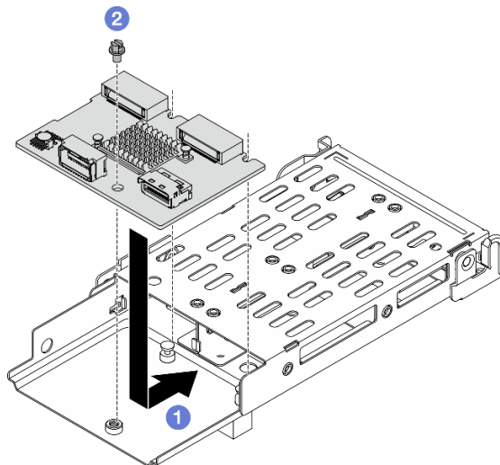
Рис. 221. Установка объединительной панели M.2
