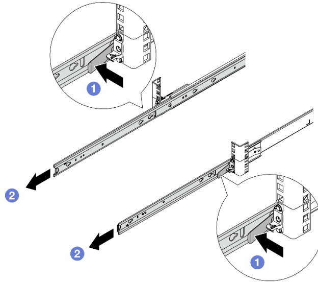
Рис. 39. Снятие внутренних направляющих
