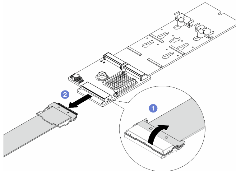
Рис. 103. Отключение кабеля M.2
