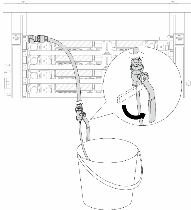
Рис. 182. Открытие клапана отводной трубки на стороне подачи
