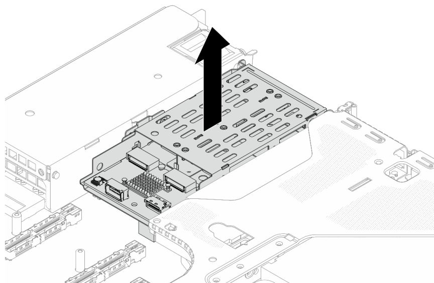
Рис. 222. Снятие отсека M.2
