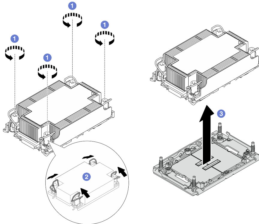
Рис. 192. Снятие модуля РНМ
