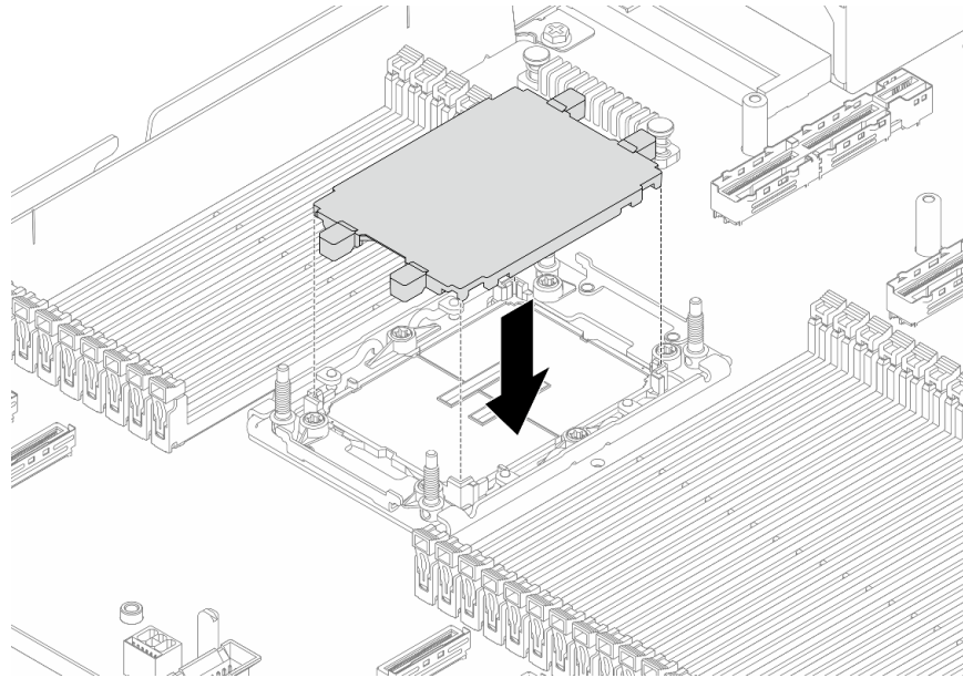
Рис. 120. Установка кожуха гнезда процессора
