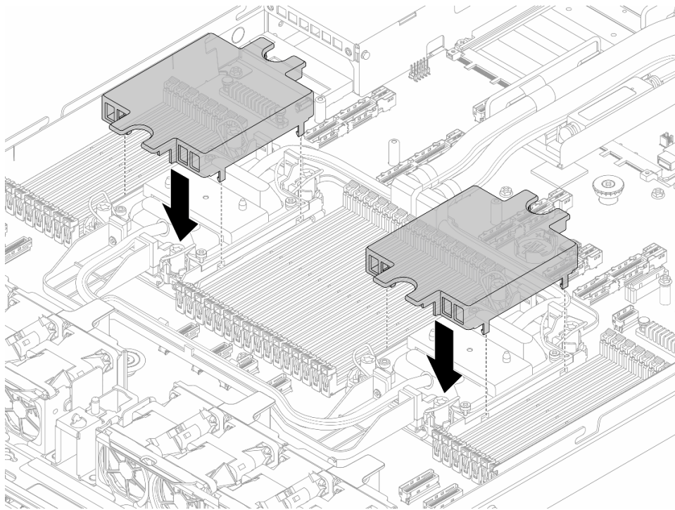
Рис. 132. Установка кожуха платы охлаждения
