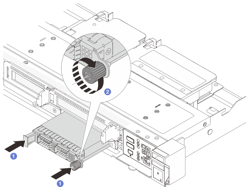
Рис. 82. Установка переднего модуля OCP
