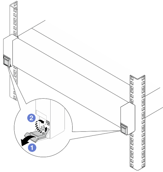
Рис. 43. Фиксация сервера на лицевой стороне стойки
