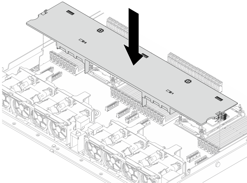
Рис. 57. Установка дефлектора
