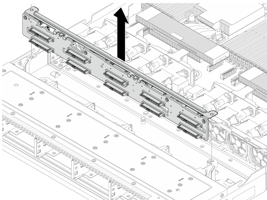
Рис. 58. Снятие объединительной панели для десяти 2,5-дюймовых оперативно заменяемых дисков
