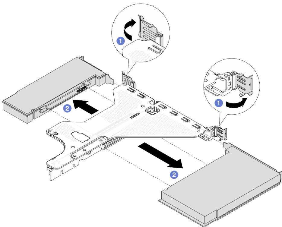
Рис. 188. Снятие адаптера PCIe с блока платы-адаптера Riser LP-FH
