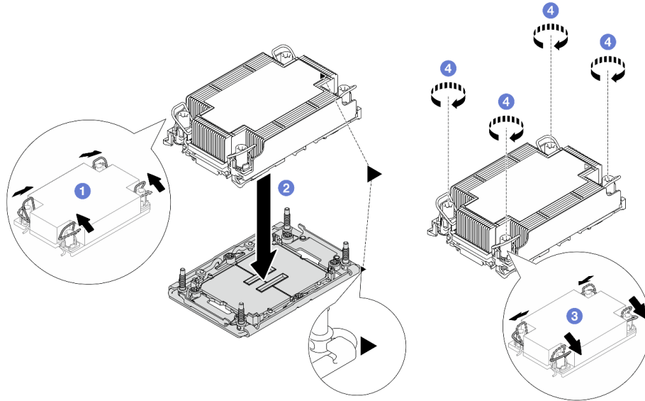
Рис. 200. Установка модуля РНМ
