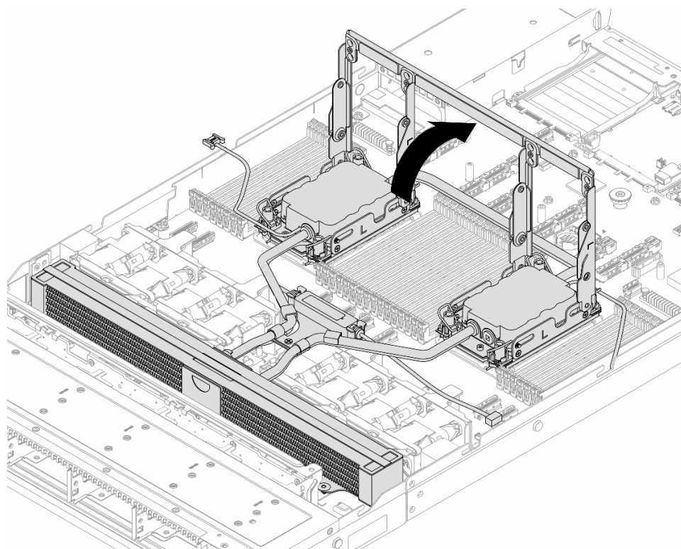
Рис. 117. Открывание ручки
