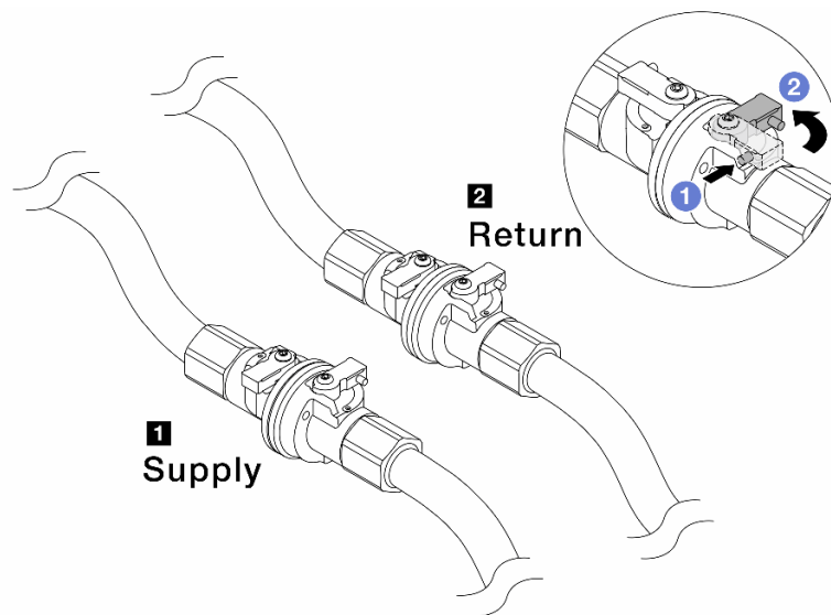
Рис. 165. Закрытие шаровых клапанов
