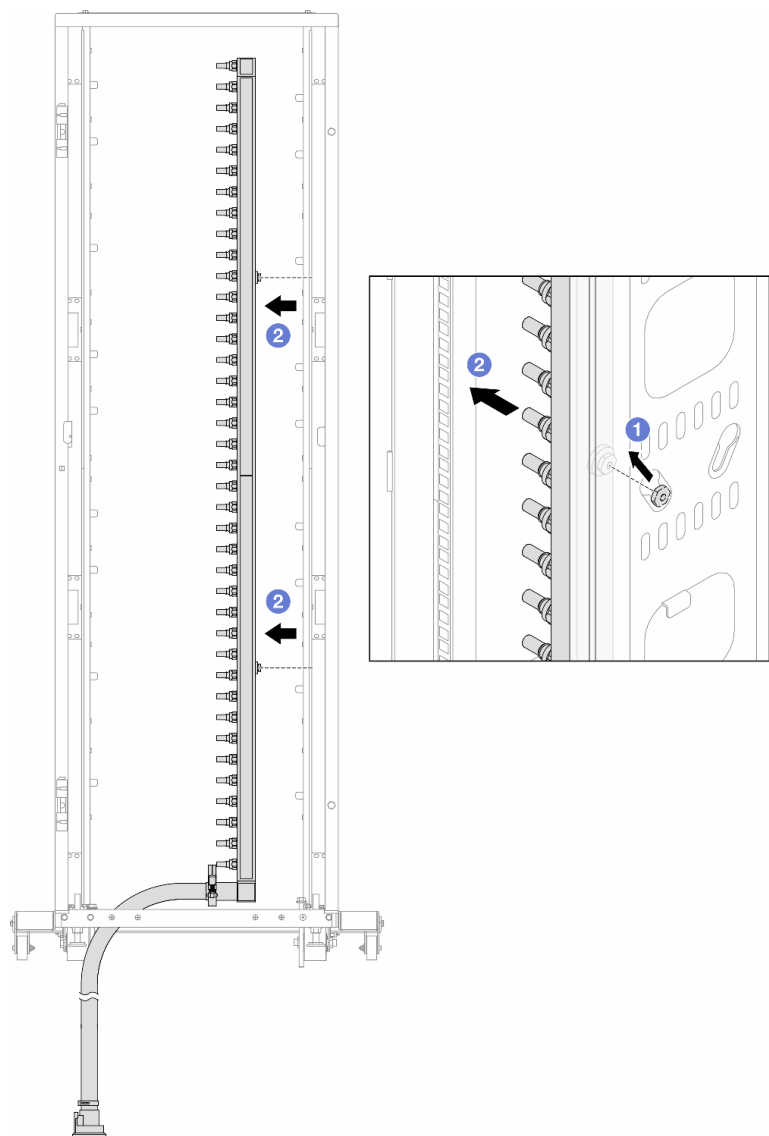
Рис. 167. Снятие коллектора
