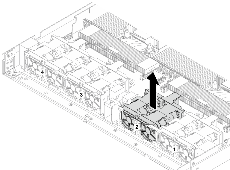
Рис. 114. Снятие блока вентиляторов 2
