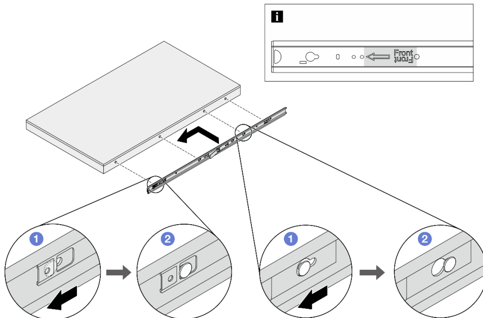
Рис. 40. Установка внутренних направляющих
