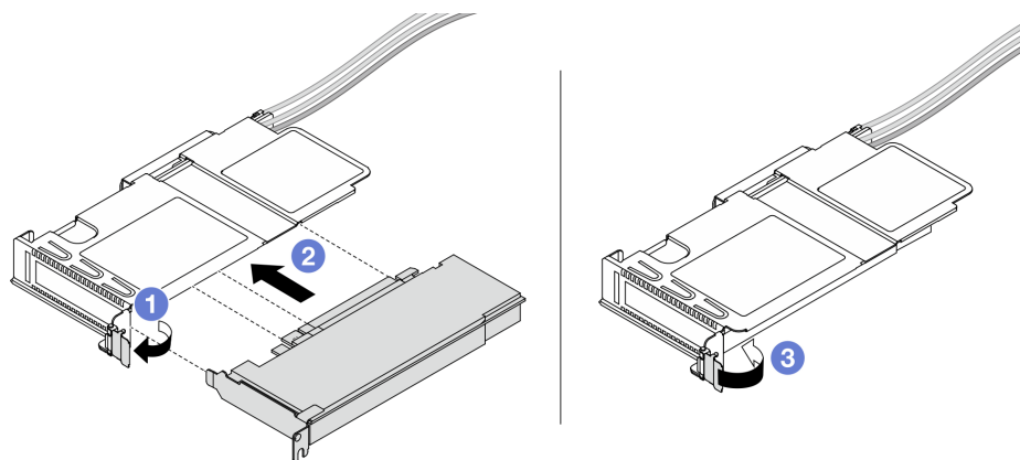
Рис. 79. Установка адаптера PCIe
