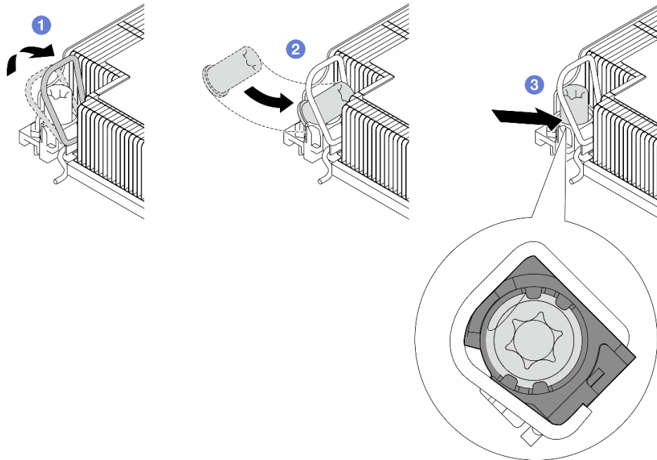
Рис. 90. Установка гайки Torx T30 в радиатор
