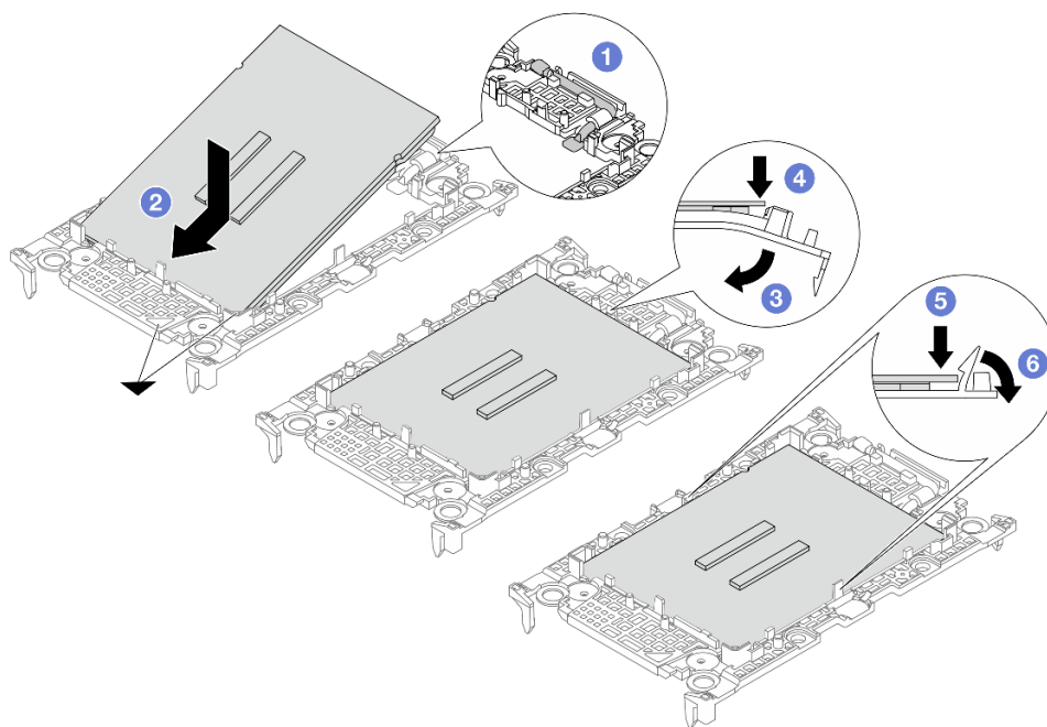
Рис. 196. Установка держателя процессора
