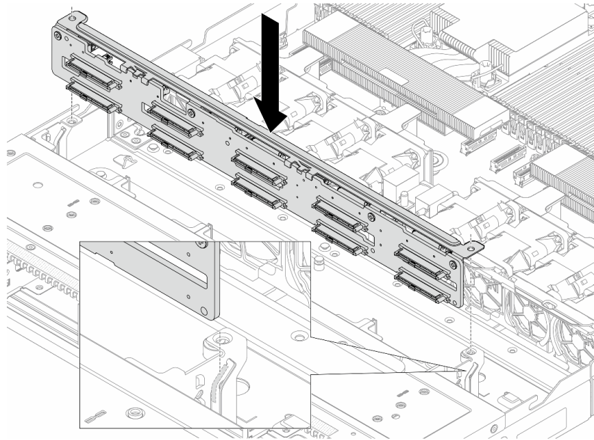
Рис. 59. Установка объединительной панели для десяти 2,5-дюймовых оперативно заменяемых дисков
