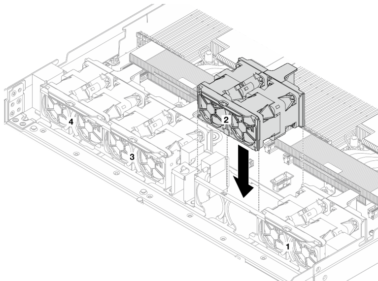
Рис. 113. Установка блока вентиляторов 2 на место
