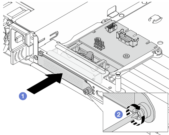
Рис. 86. Установка задней карты интерпозера OCP
