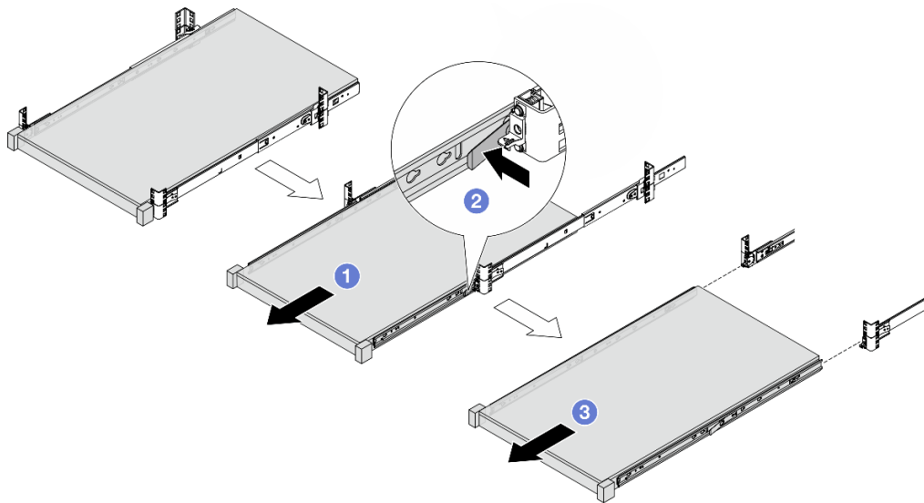
Рис. 37. Снятие сервера
