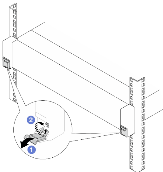
Рис. 54. Фиксация сервера на лицевой стороне стойки
