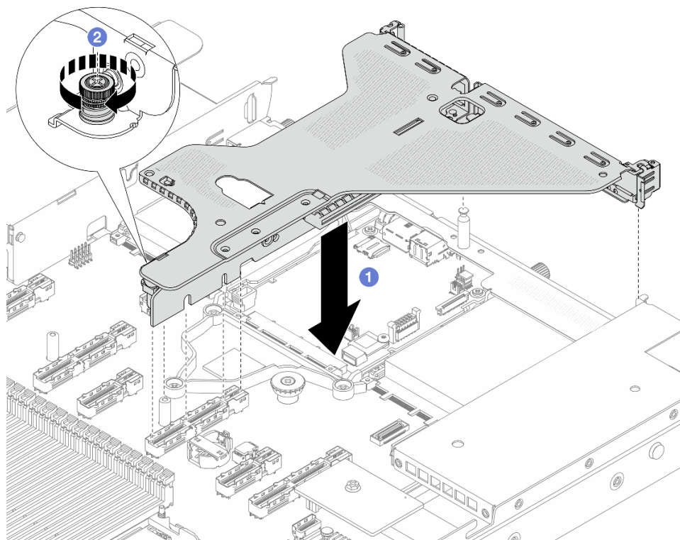
Рис. 266. Установка блока платы-адаптера Riser
