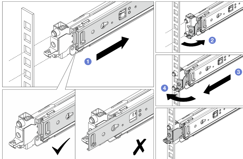
Рис. 34. Установка передних крепежных контактов
