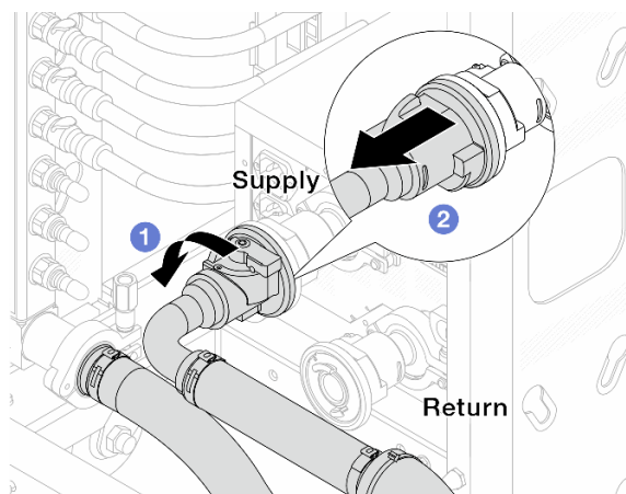
Рис. 144. Снятие комплекта соединений
