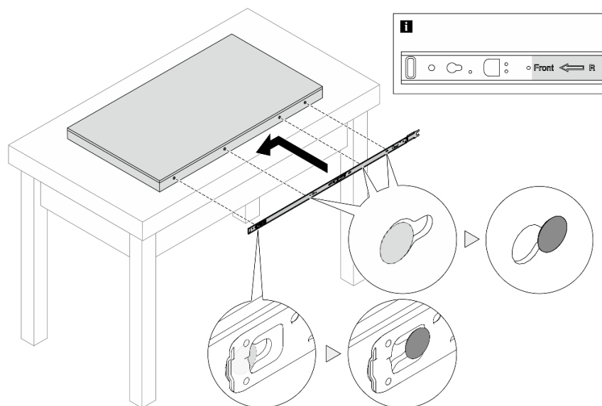
Рис. 50. Установка внутренних направляющих
