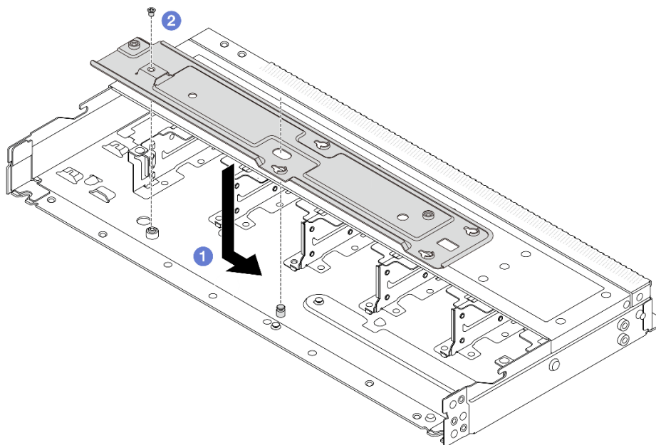
Рис. 119. Установка лотка радиатора
