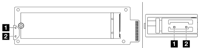
Рис. 302. Светодиодные индикаторы заднего интерпозера M.2
