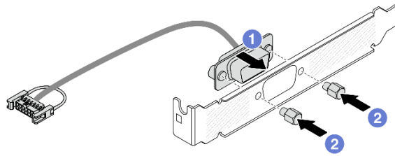
Рис. 275. Сборка модуля последовательного порта
