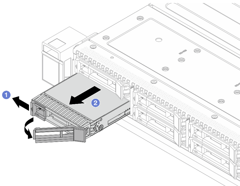
Рис. 91. Снятие оперативно заменяемого диска
