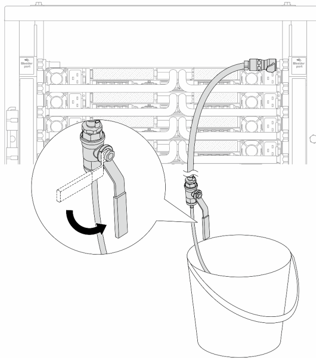
Рис. 181. Открытие клапана отводной трубки на стороне возврата
