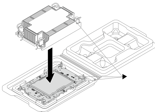
Рис. 198. Сборка модуля процессора с радиатором (PHM), когда процессор находится в транспортировочном лотке
