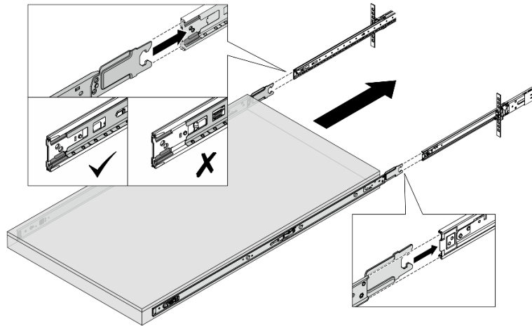
Рис. 52. Взаимоблокировка направляющих
