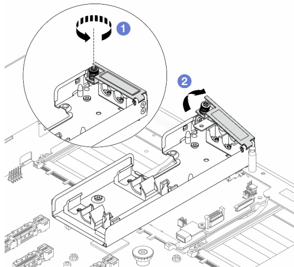
Рис. 127. Открывание кожуха держателя
