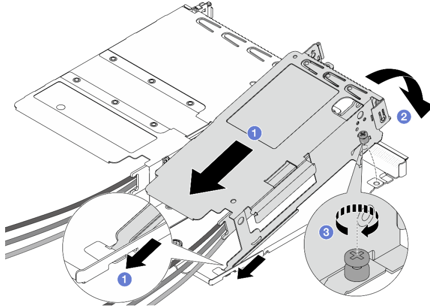
Рис. 80. Сборка двух отсеков плат-адаптеров Riser
