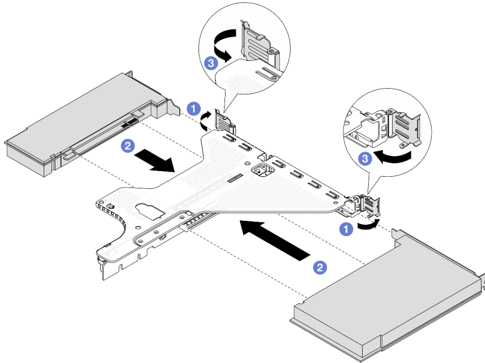
Рис. 189. Установка адаптера PCIe в блок платы-адаптера Riser LP-FH
