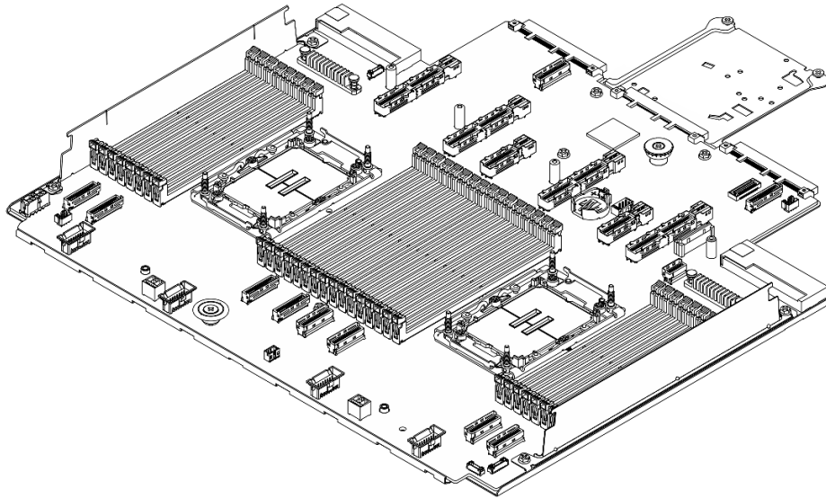
Рис. 282. Процессорная плата
