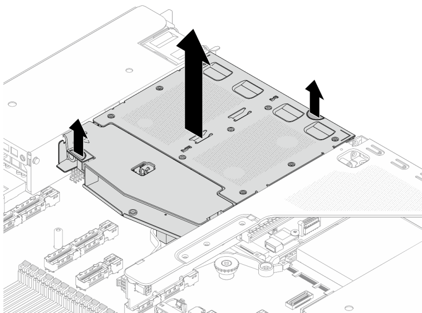
Рис. 204. Снятие заднего отсека для 2,5-дюймовых дисков
