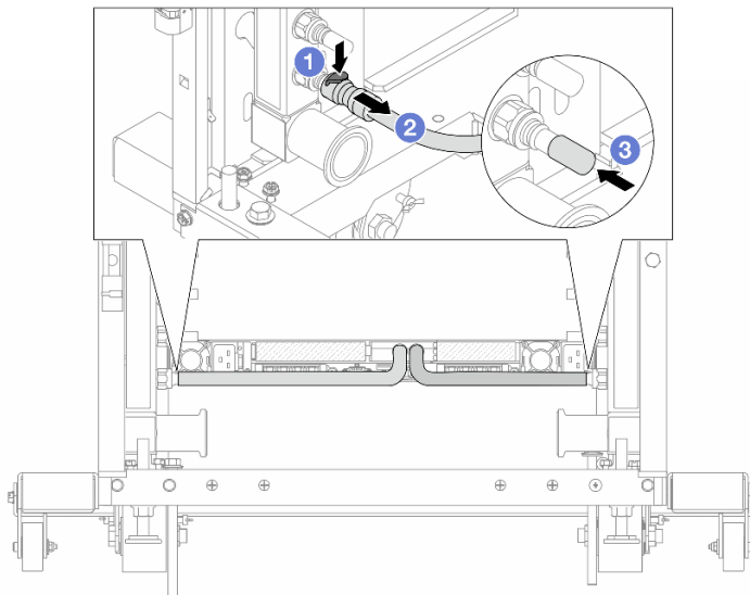
Рис. 143. Отсоединение быстроразъемного соединителя
