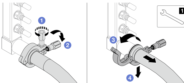
Рис. 150. Отделение коллектора от комплекта соединений
