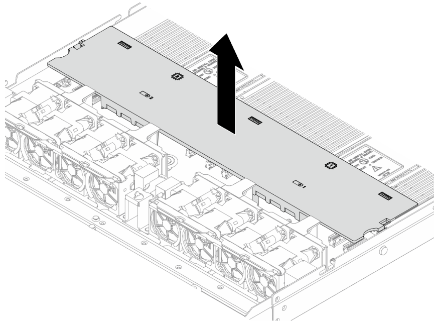
Рис. 56. Снятие дефлектора
