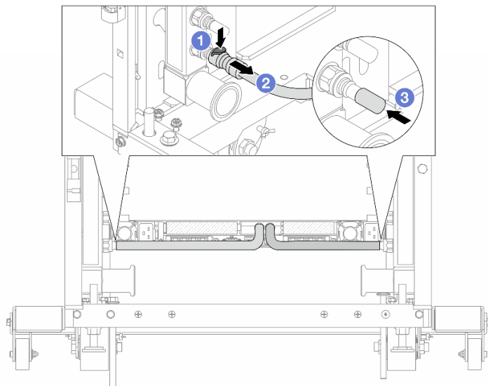
Рис. 166. Отсоединение быстроразъемного соединителя
