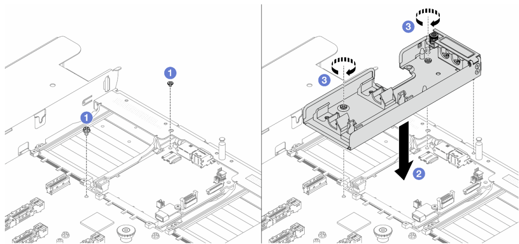
Рис. 126. Установка держателя шланга
