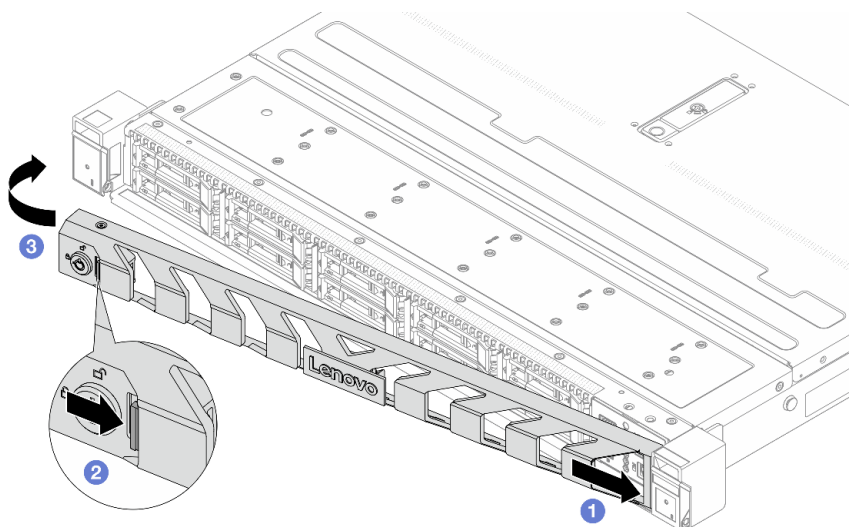
Рис. 270. Установка защитной панели
