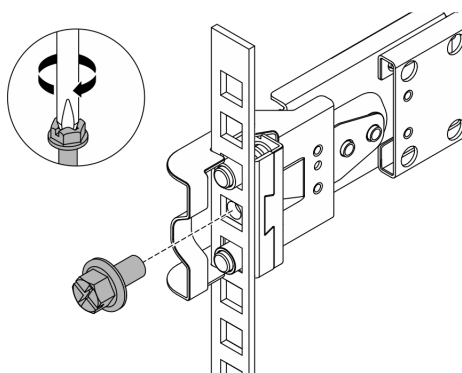
Рис. 55. Фиксация сервера на задней стороне стойки
