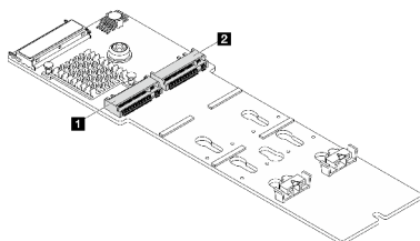
Рис. 107. Гнездо для диска M.2
