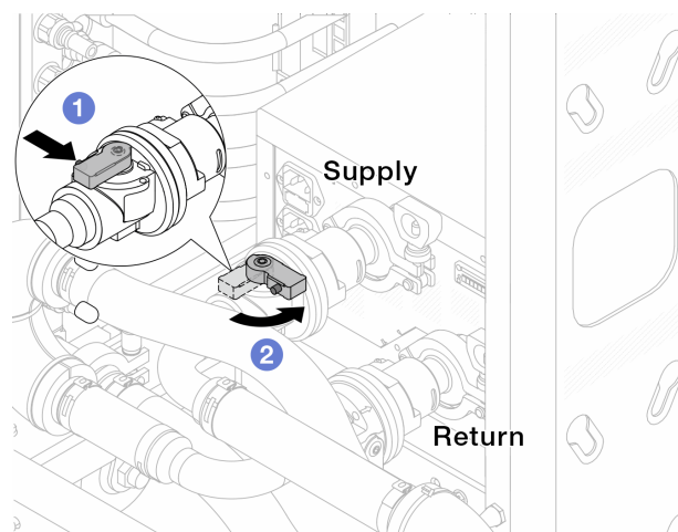
Рис. 142. Закрытие шаровых клапанов
