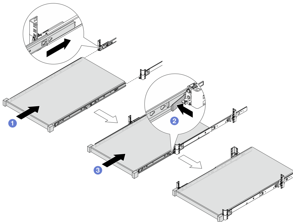
Рис. 42. Установка сервера
