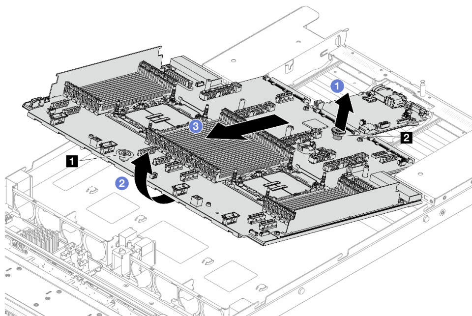
Рис. 281. Снятие блока материнской платы
