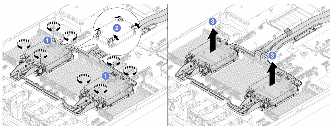
Рис. 124. Снятие компонента «модуль NeptCore»
