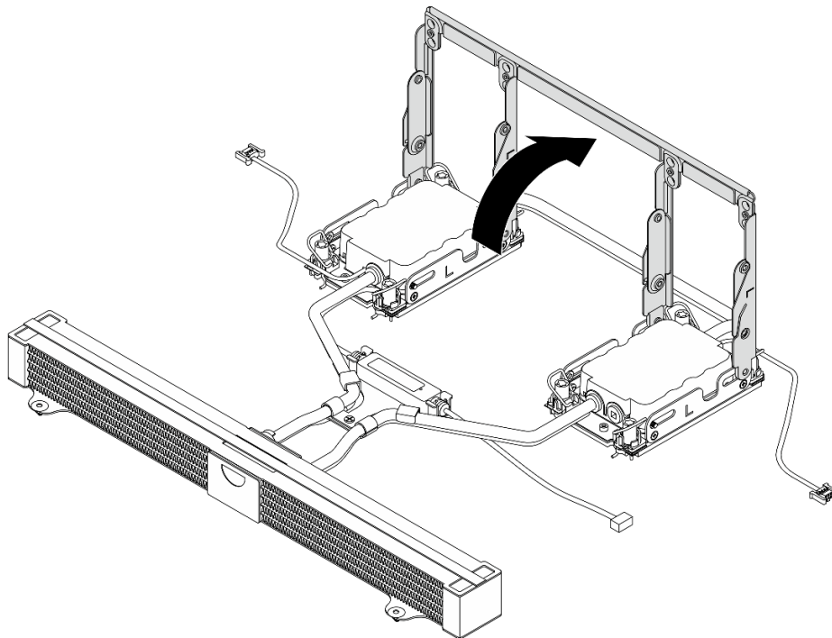
Рис. 121. Открывание ручки
