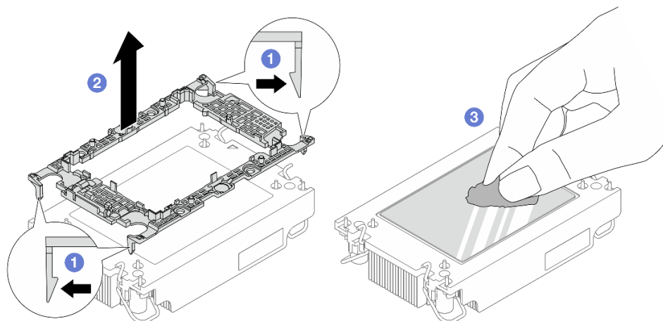
Рис. 194. Снятие держателя процессора с радиатора
