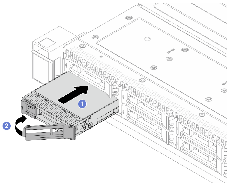
Рис. 94. Установка оперативно заменяемого диска
