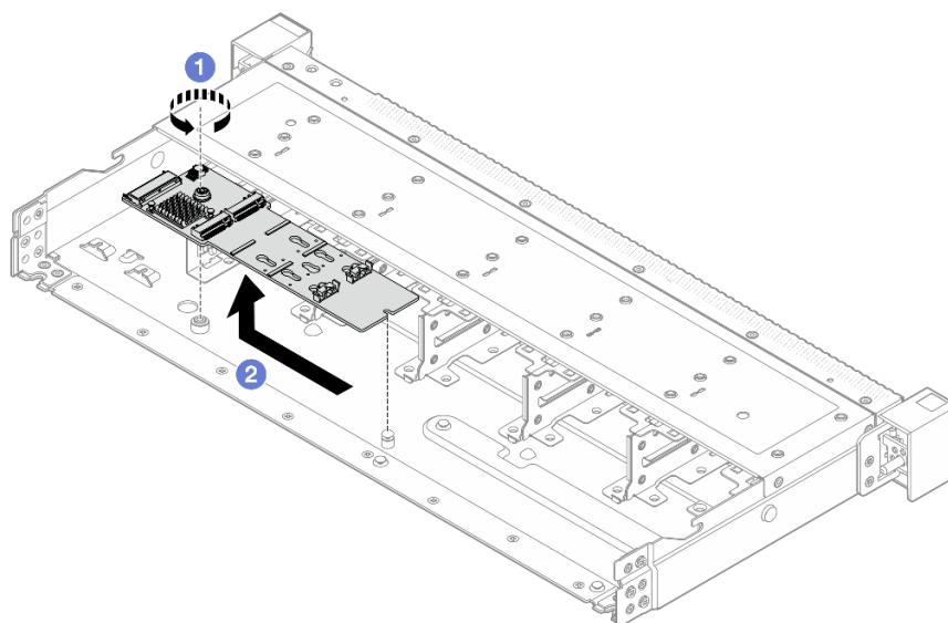
Рис. 105. Снятие модуля M.2
