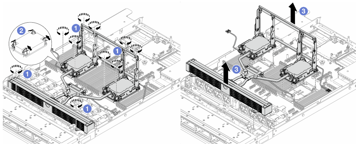
Рис. 118. Снятие компонента «модуль NeptAir»
