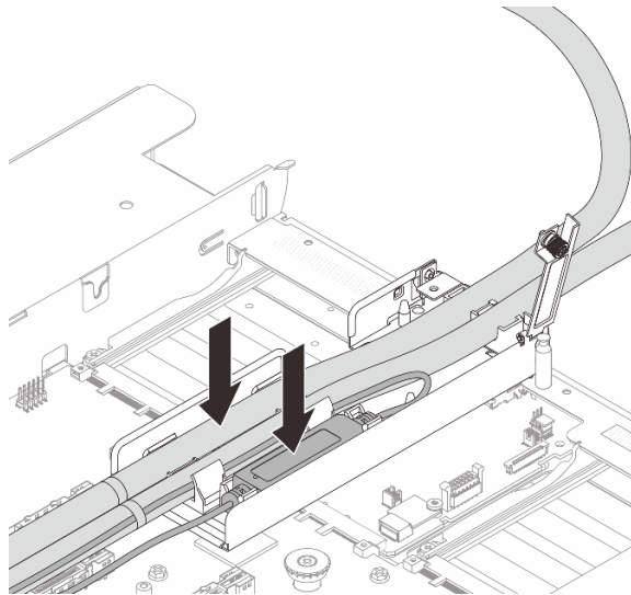
Рис. 133. Размещение шлангов и модуля
