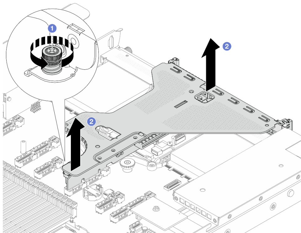
Рис. 263. Снятие блока платы-адаптера Riser
