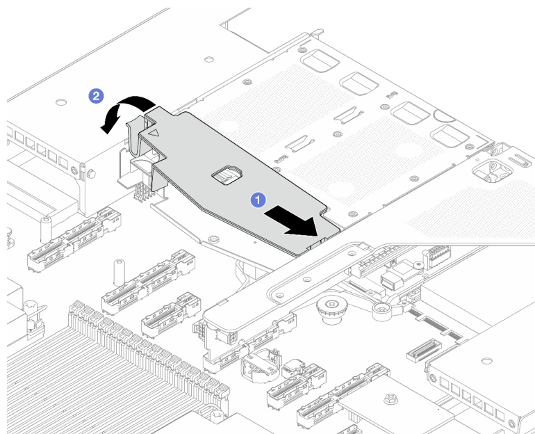
Рис. 207. Установка дефлектора
