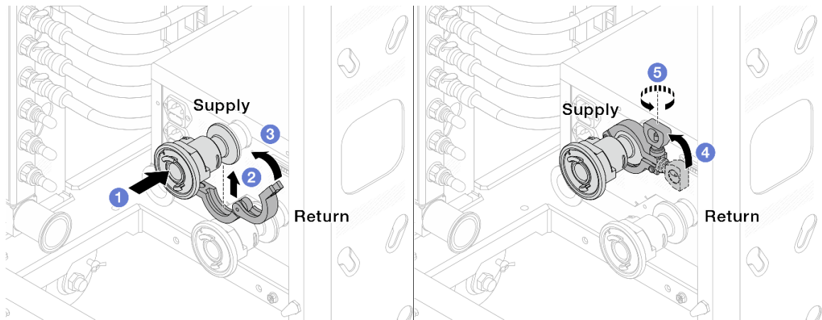
Рис. 153. Установка шаровых клапанов
