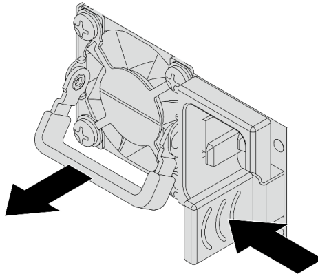
Рис. 97. Снятие оперативно заменяемого блока питания
