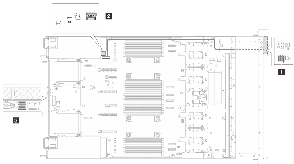
Рис. 307. Обзор USB-портов
