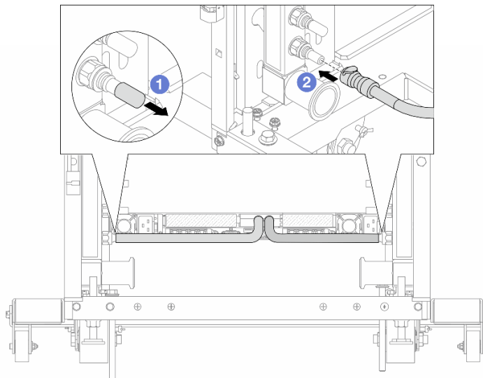
Рис. 174. Установка быстроразъемного соединителя
