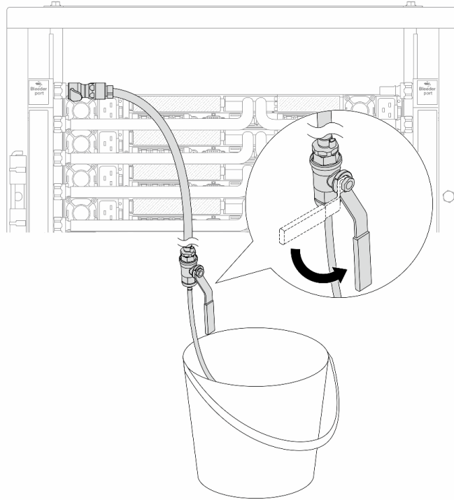
Рис. 161. Открытие клапана отводной трубки на стороне подачи
