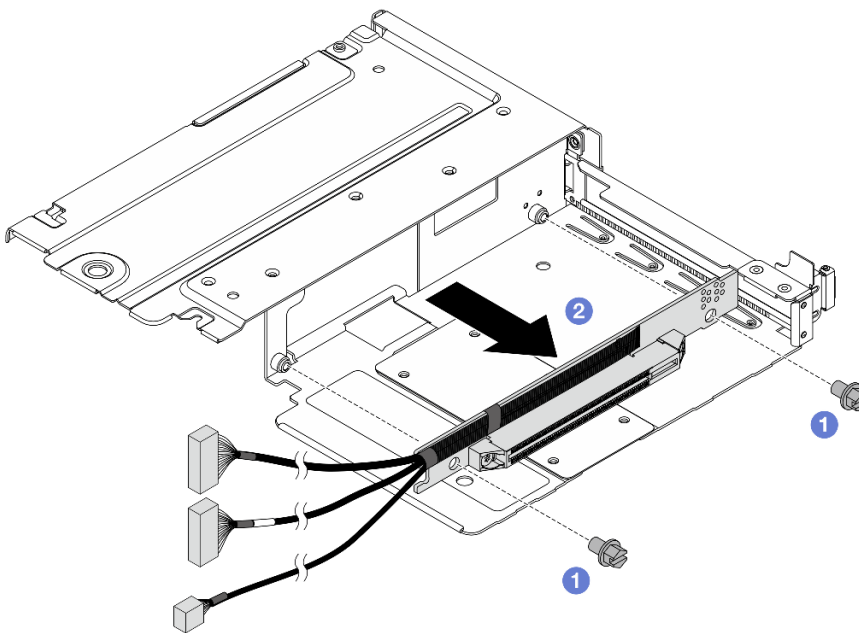
Рис. 76. Снятие платы-адаптера Riser с отсека максимальной высоты
