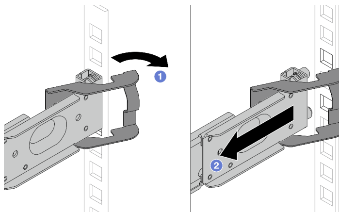
Рис. 30. Снятие направляющей сзади
