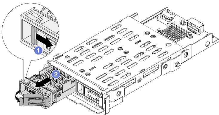
Рис. 218. Снятие заднего блока диска M.2
