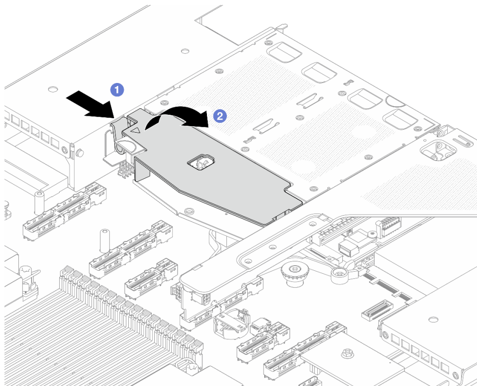
Рис. 205. Снятие дефлектора
