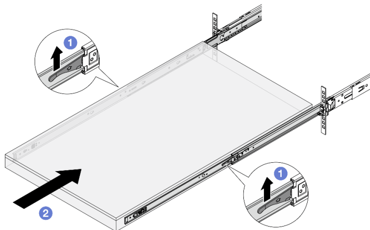
Рис. 53. Блокировка направляющих и установка сервера
