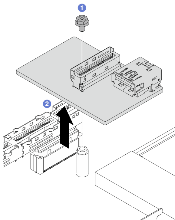
Рис. 288. Снятие платы ввода-вывода USB
