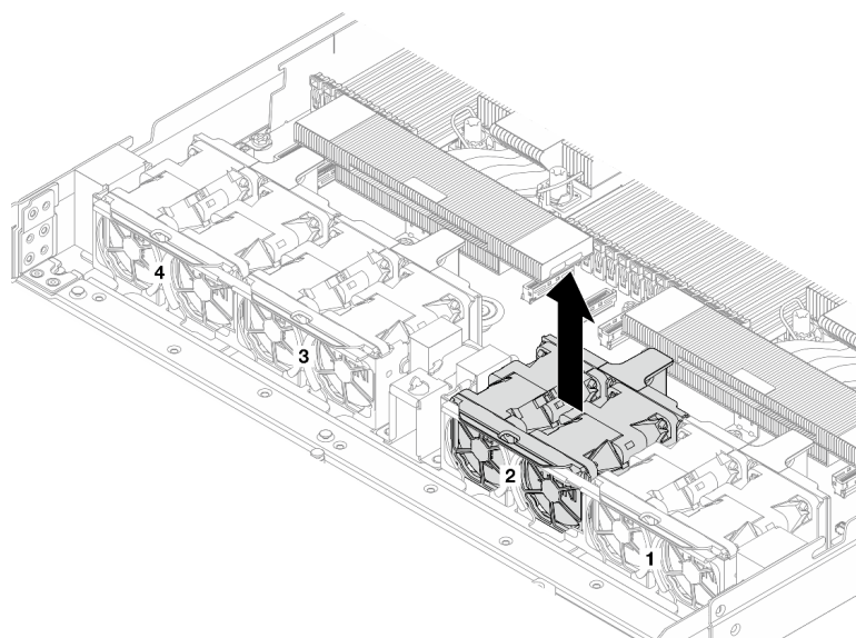
Рис. 111. Снятие блока вентиляторов 2
