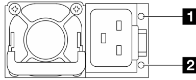
Рис. 299. Светодиодные индикаторы на модуле блока питания CRPS Premium
