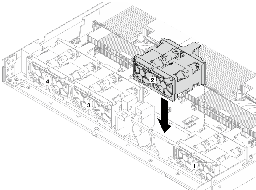
Рис. 285. Установка блока вентиляторов компьютера
