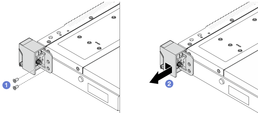
Рис. 202. Снятие защелки стойки
