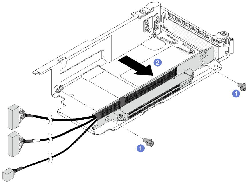
Рис. 75. Снятие платы-адаптера Riser с низкопрофильного отсека
