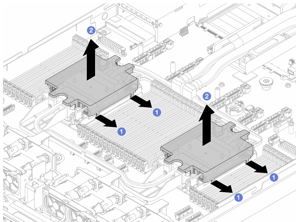
Рис. 306. Снятие кожуха платы охлаждения
