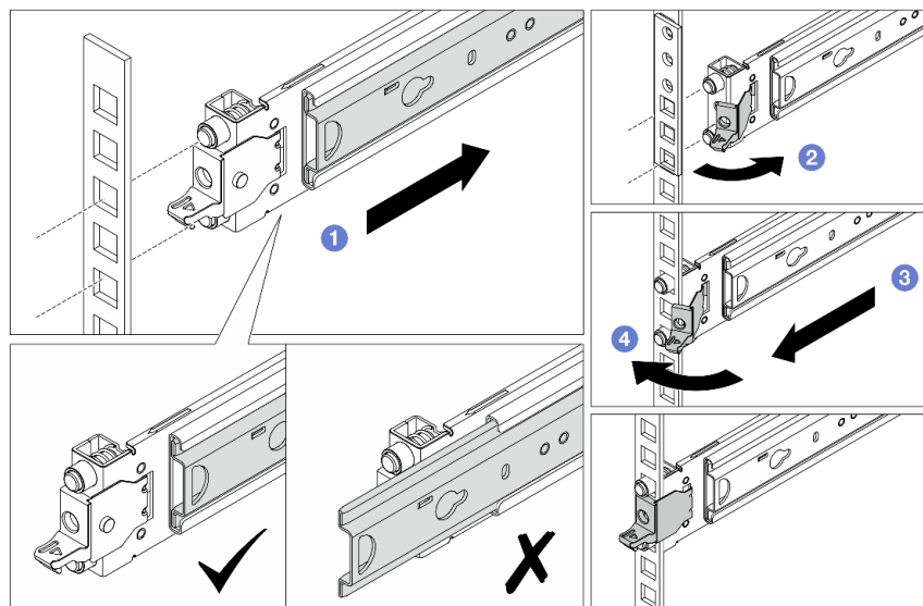
Рис. 32. Установка передних крепежных контактов
