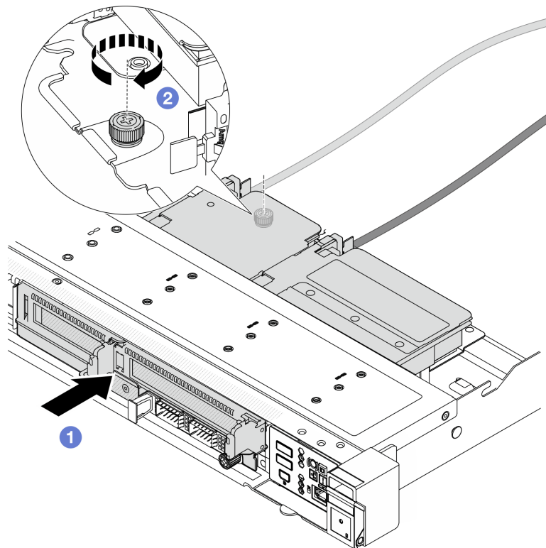
Рис. 72. Установка переднего отсека платы-адаптера Riser
