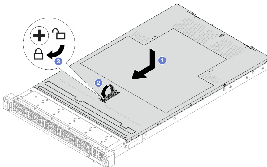
Рис. 287. Установка верхнего кожуха
