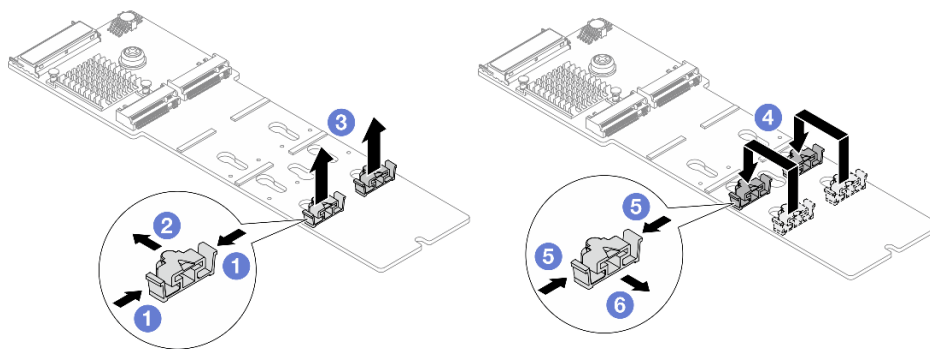
Рис. 106. Регулировка фиксатора M.2
