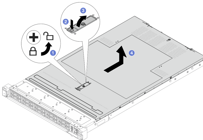
Рис. 286. Снятие верхнего кожуха
