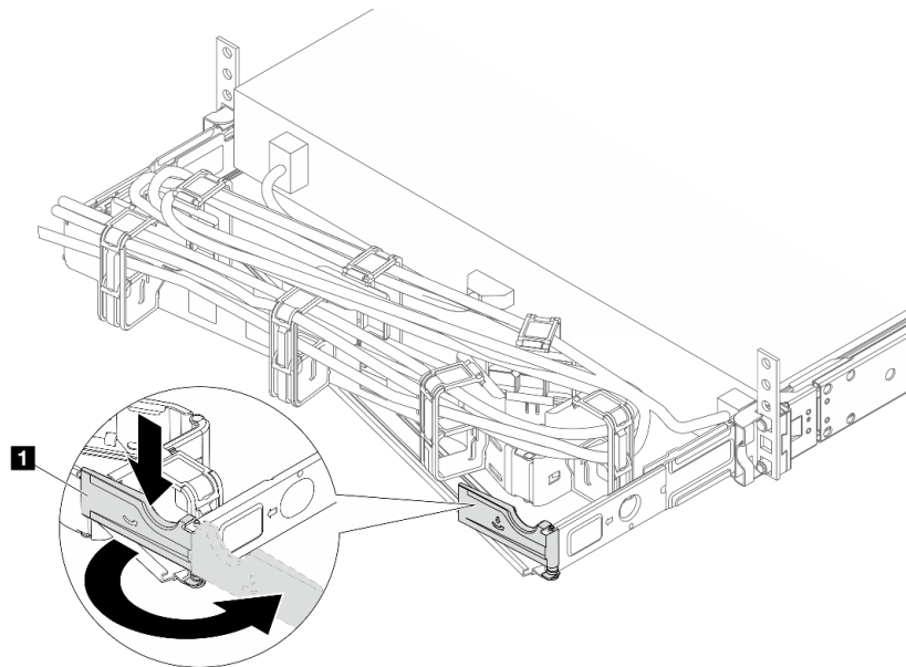
Рис. 95. Регулировка правой стороны
