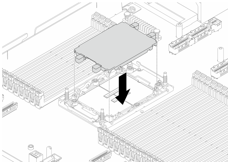
Рис. 129. Установка кожуха гнезда процессора
