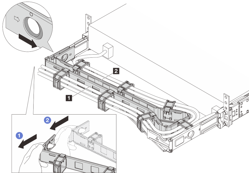
Рис. 96. Снятие левой стороны
