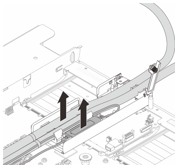
Рис. 123. Отсоединение шлангов и модуля
