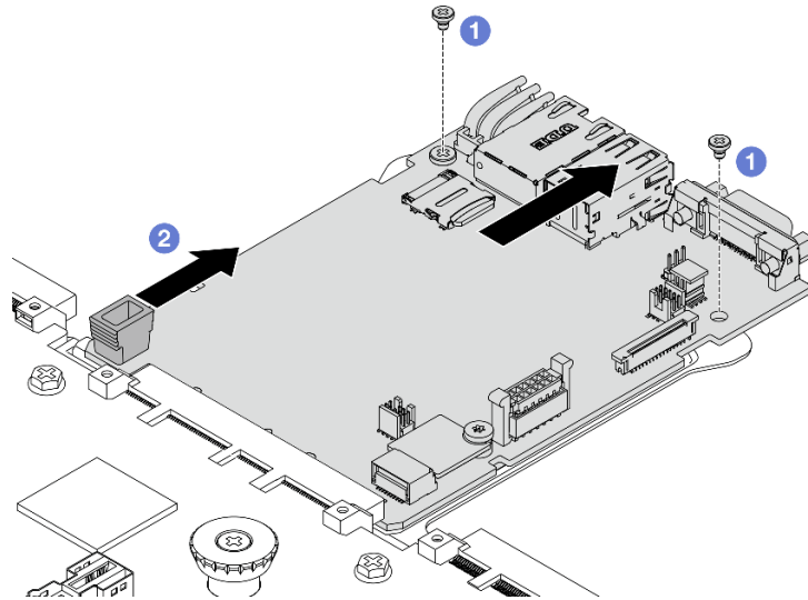
Рис. 279. Снятие системной платы ввода-вывода
