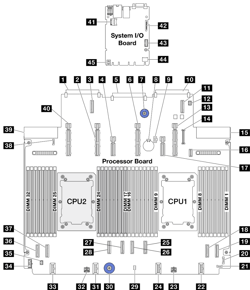
Рис. 292. Разъемы блока материнской платы
