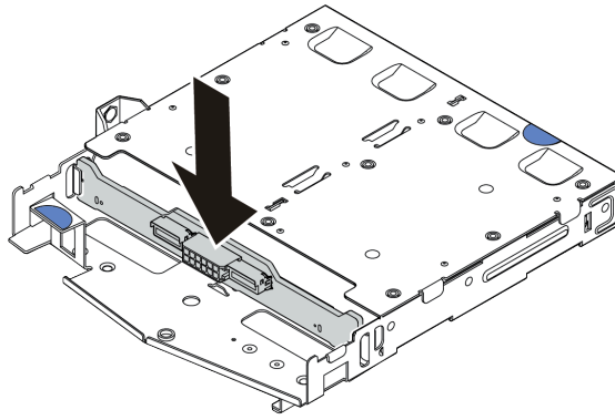
Рис. 62. Установка задней объединительной панели
