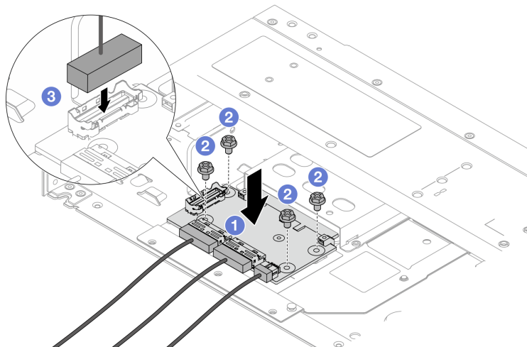
Рис. 84. Установка передней карты интерпозера OCP
