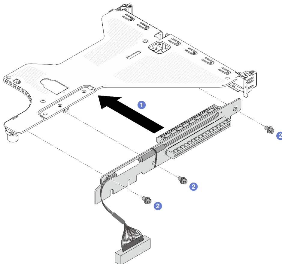
Рис. 265. Установка платы-адаптера Riser
