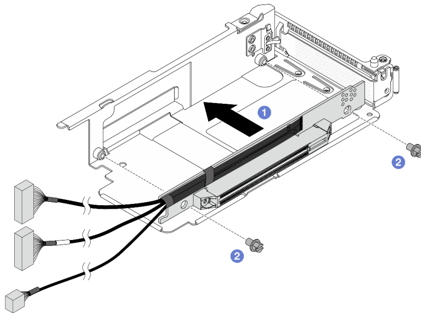
Рис. 77. Установка платы-адаптера Riser в низкопрофильный отсек
