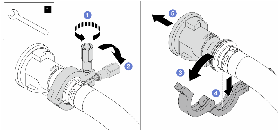
Рис. 152. Отделение шаровых клапанов
