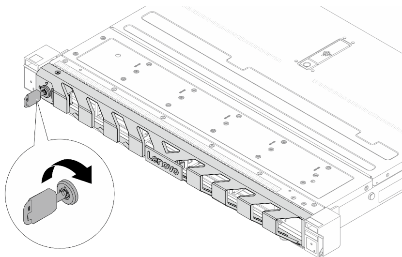
Рис. 267. Разблокирование защитной панели
