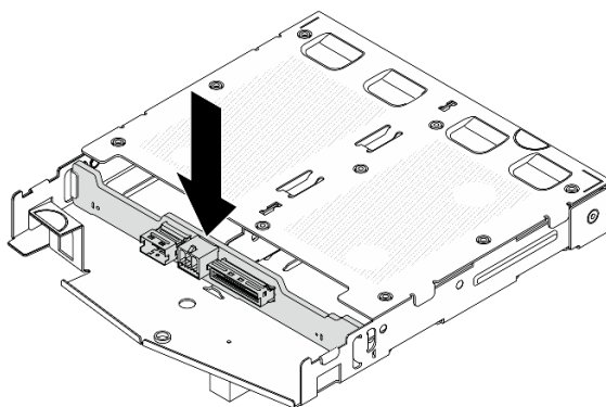
Рис. 206. Установка задней объединительной панели
