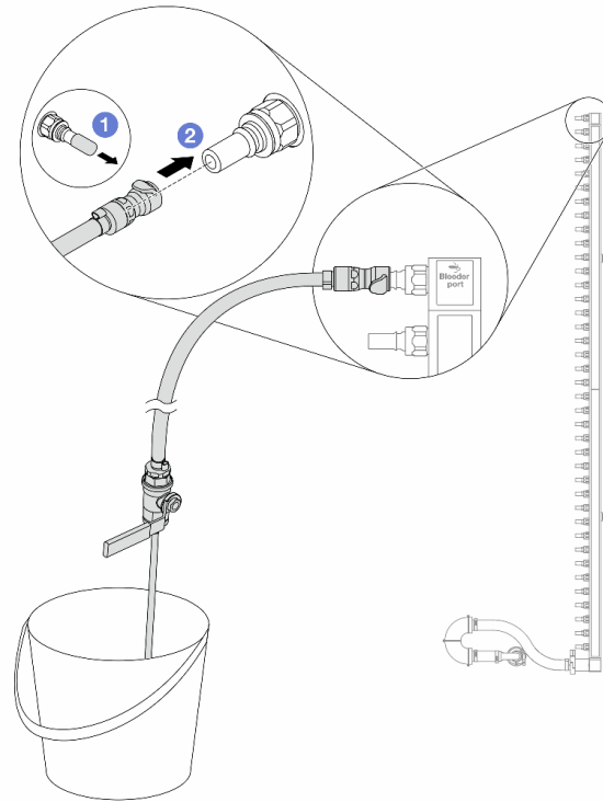
Рис. 148. Установка комплекта отводной трубки на стороне возврата
