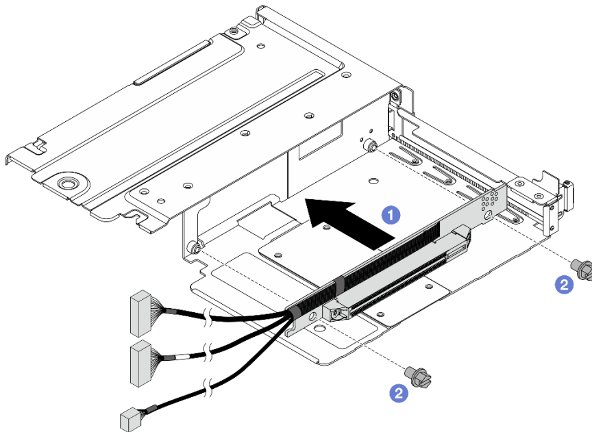
Рис. 78. Установка платы-адаптера Riser в отсек максимальной высоты
