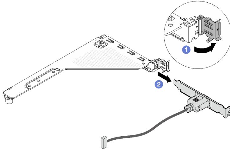
Рис. 273. Снятие скобы платы-адаптера Riser
