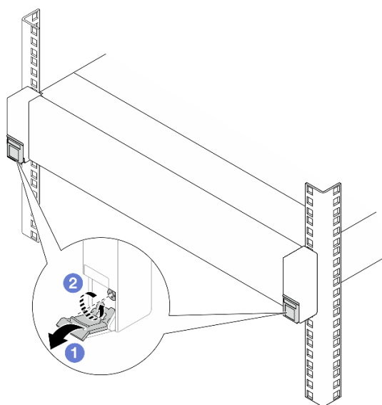
Рис. 35. Ослабление винтов в защелках стойки
