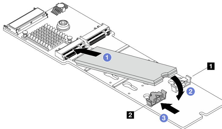
Рис. 109. Установка диска M.2
