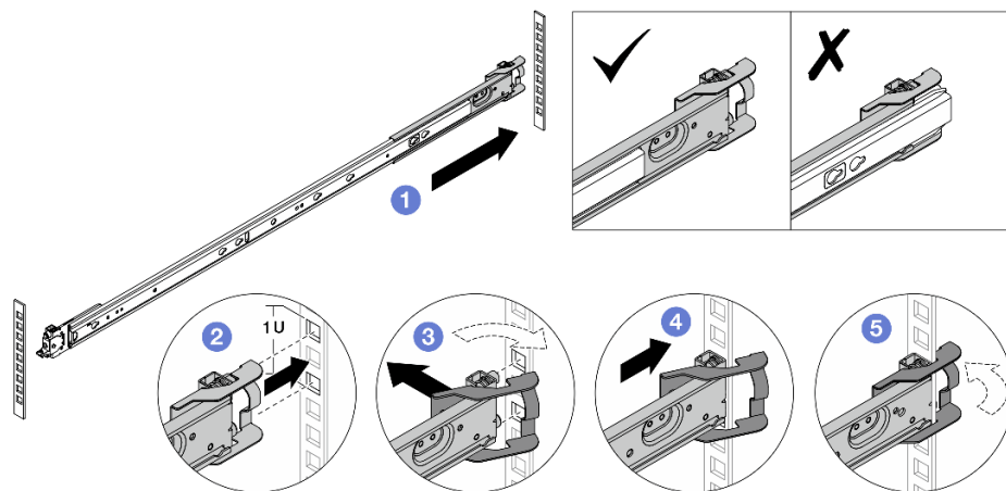
Рис. 31. Установка задних крепежных контактов
