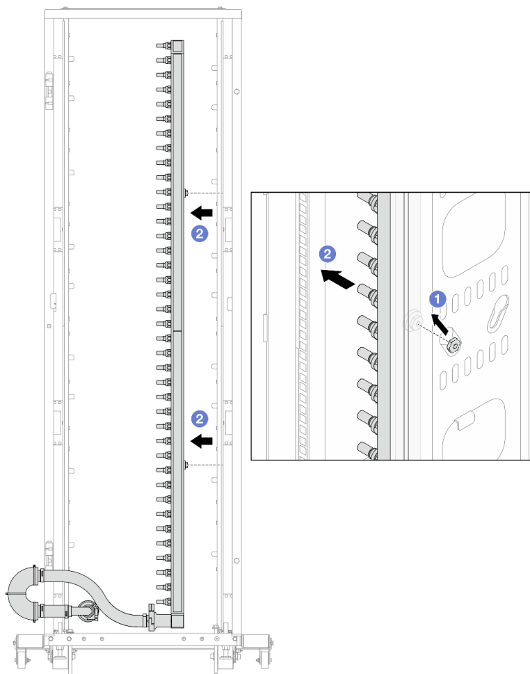
Рис. 145. Снятие коллектора
