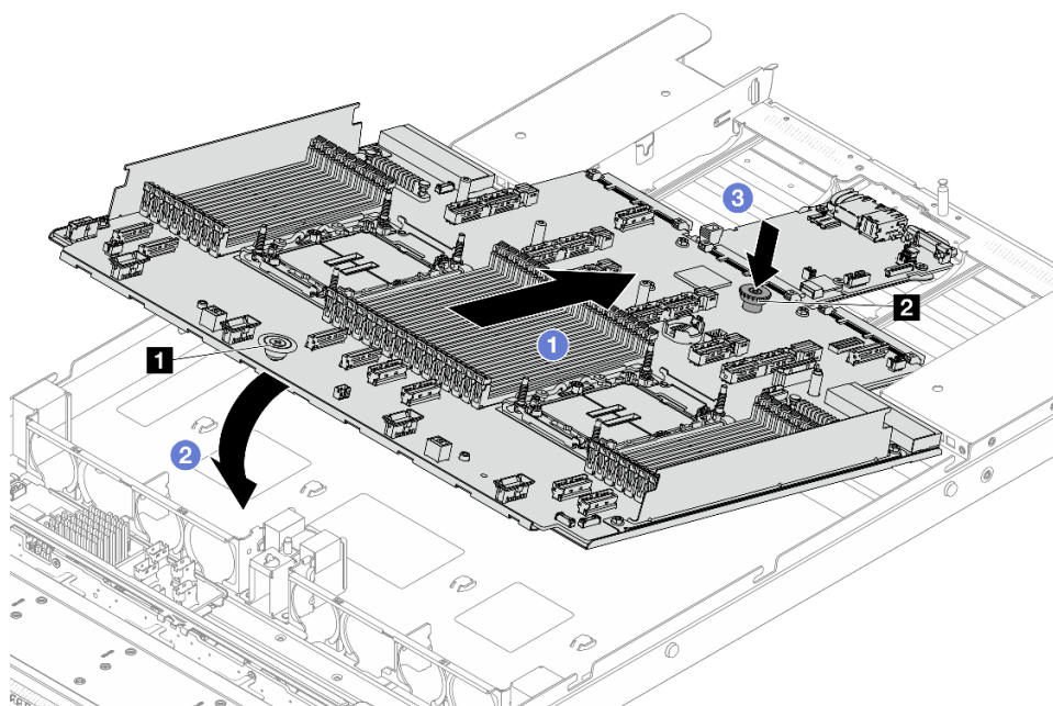
Рис. 283. Установка блока материнской платы
