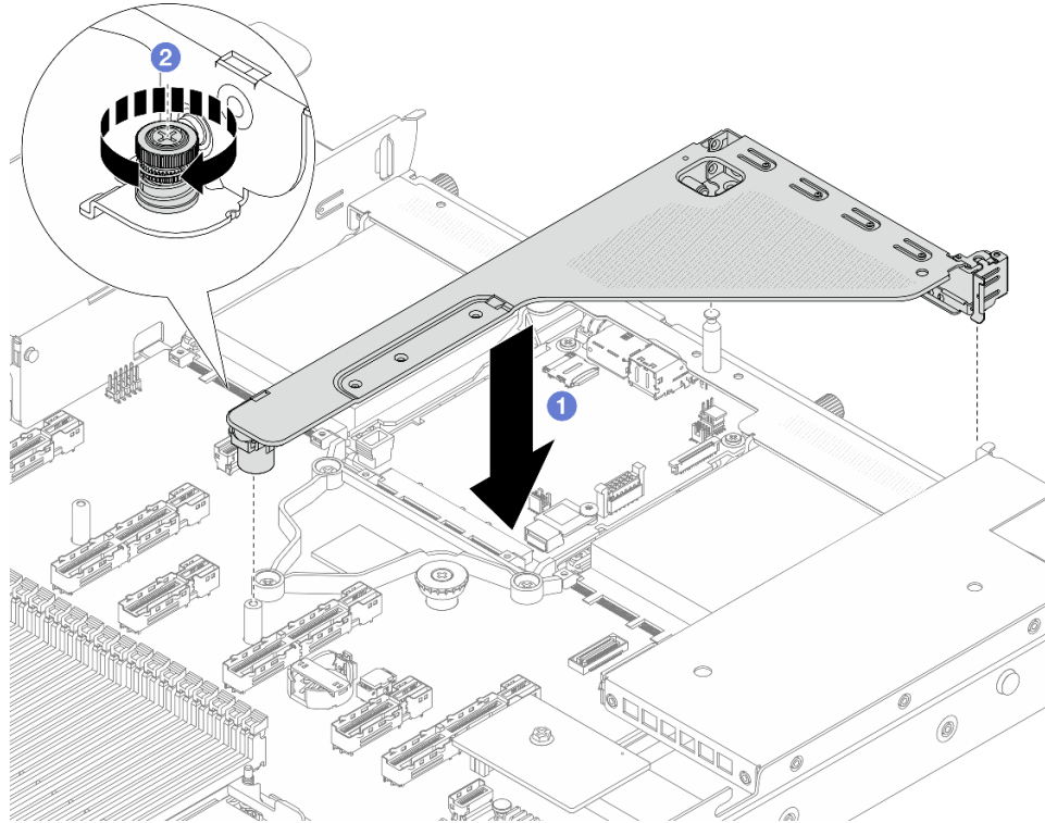
Рис. 277. Установка блока платы-адаптера Riser
