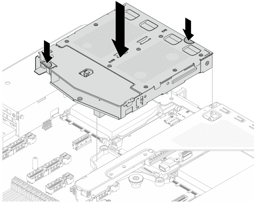
Рис. 208. Установка заднего отсека для 2,5-дюймовых дисков
