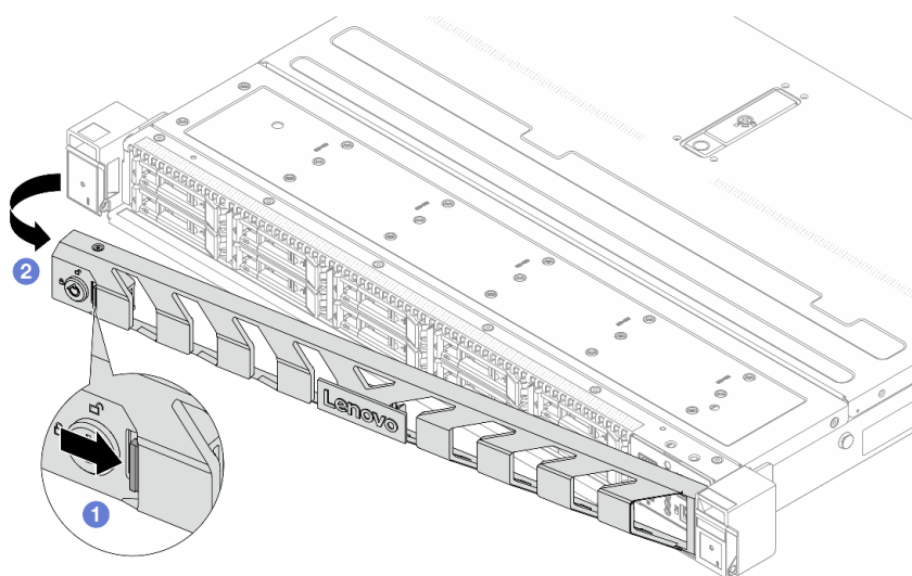
Рис. 268. Снятие защитной панели
