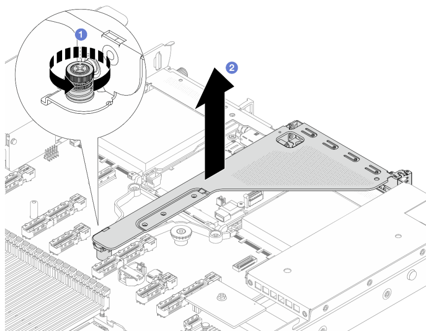
Рис. 272. Снятие скобы платы-адаптера Riser
