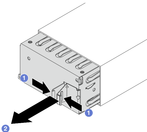
Рис. 100. Снятие заглушки оперативно заменяемого модуля блока питания
