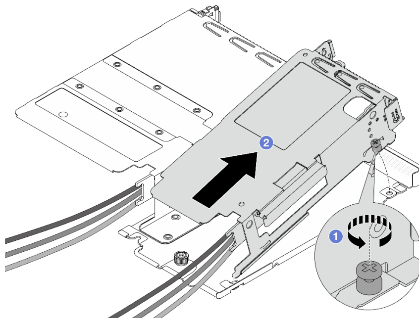
Рис. 73. Отделение двух отсеков
