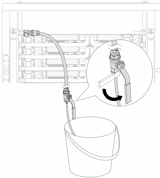
图 179. 打开供给端的泄放阀门
