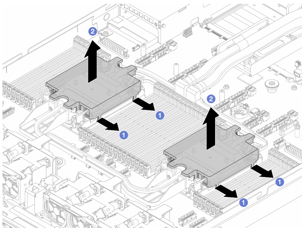
图 293. 卸下冷却板外盖
