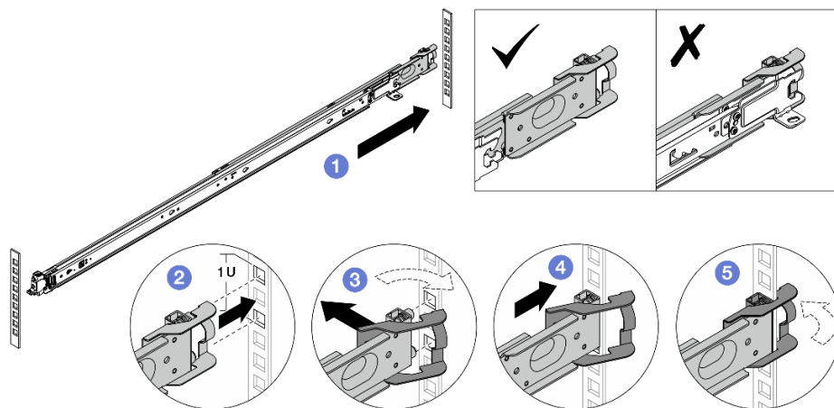
图 33. 安装背面安装销
