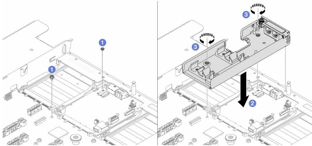
图 123. 安装软管夹持器
