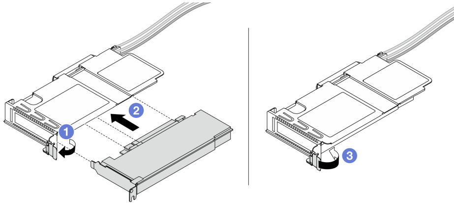
图 79. 安装 PCIe 适配器
