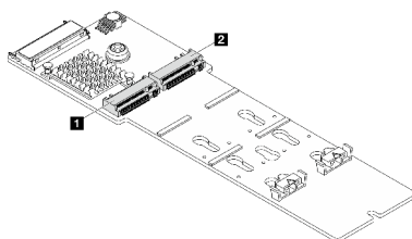
图 105. M.2 硬盘插槽
