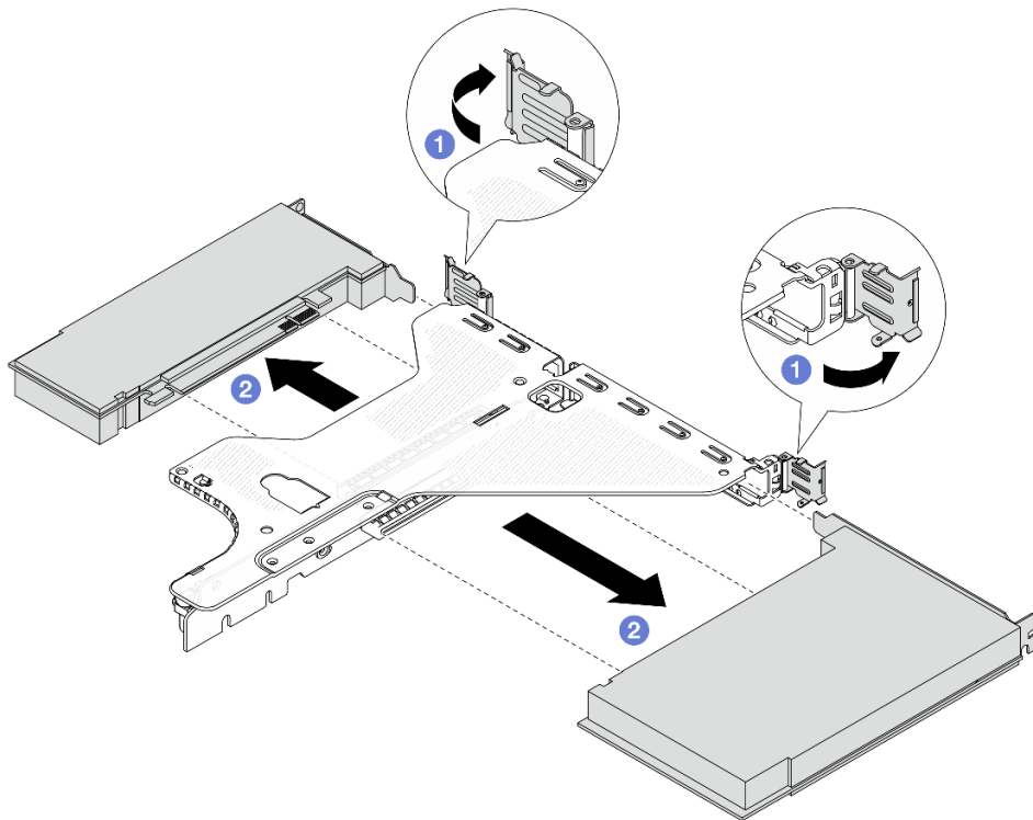
图 185. 从 LP-FH 转接卡组合件上卸下 PCIe 适配器
