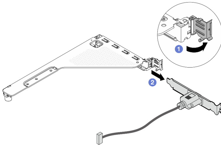
图 271. 卸下转接卡支架
