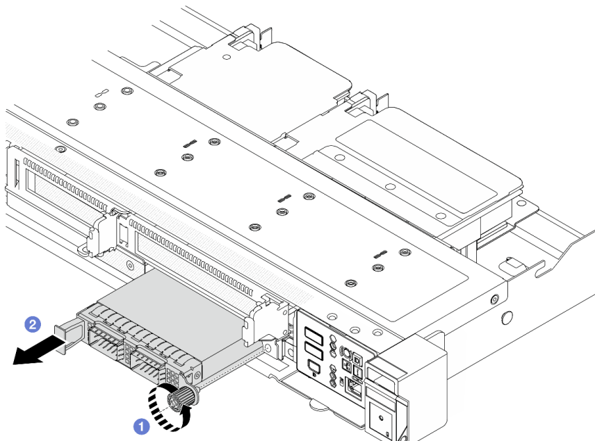
图 81. 卸下正面 OCP 模块
