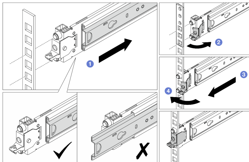
图 32. 安装正面安装销
