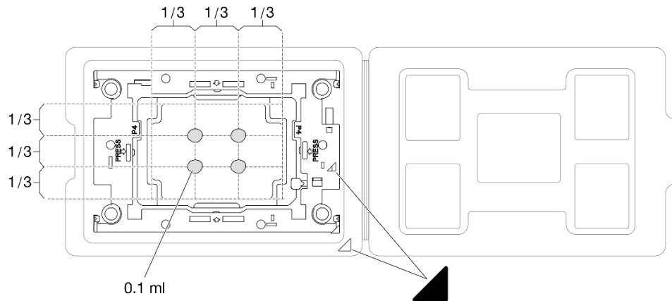
图 194. 为装运托盘中的处理器涂抹导热油脂
