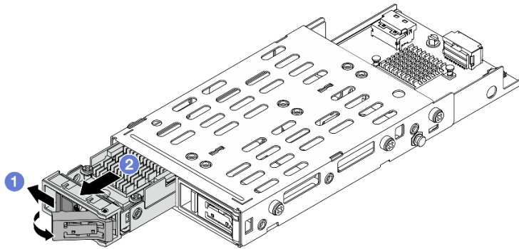
图 214. 卸下背面 M.2 硬盘组合件
