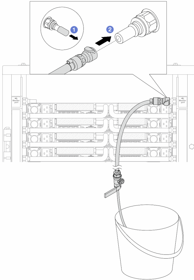
图 159. 将排气套件安装到回流端
