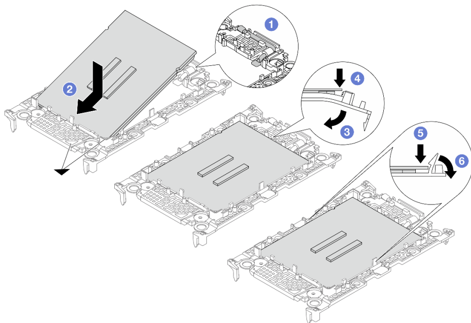
图 193. 安装处理器支架
