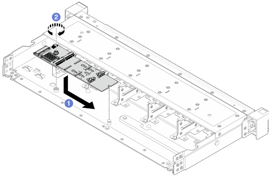
图 106. 安装 M.2 背板
