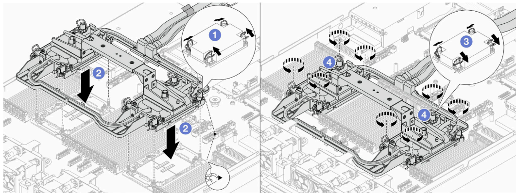
图 127. 安装 NeptCore 模块
