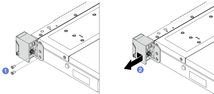
图 199. 卸下机架滑锁
