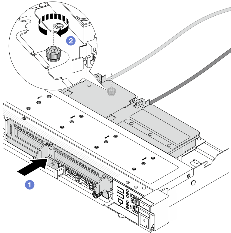
图 72. 安装正面转接卡架
