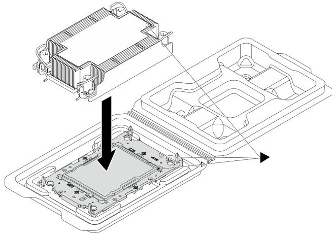
图 195. 在装运托盘中组装 PHM 和处理器
