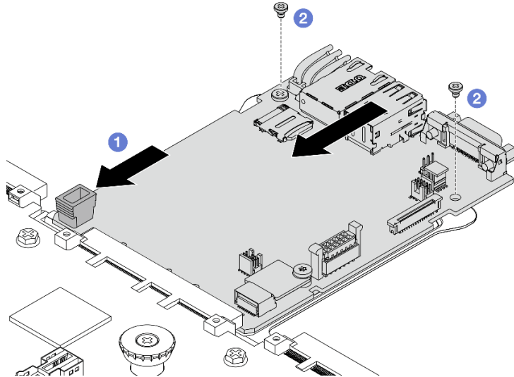
图 278. 安装系统 I/O 板
