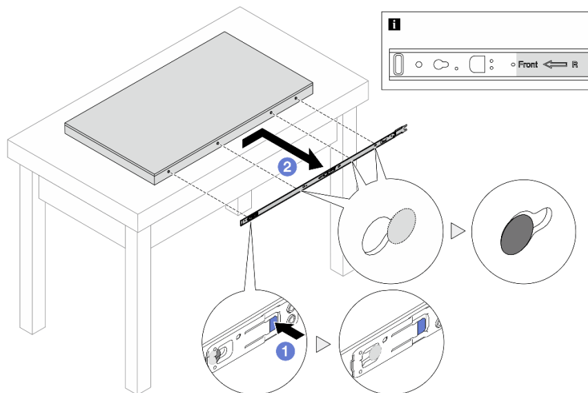
图 48. 卸下内侧导轨
