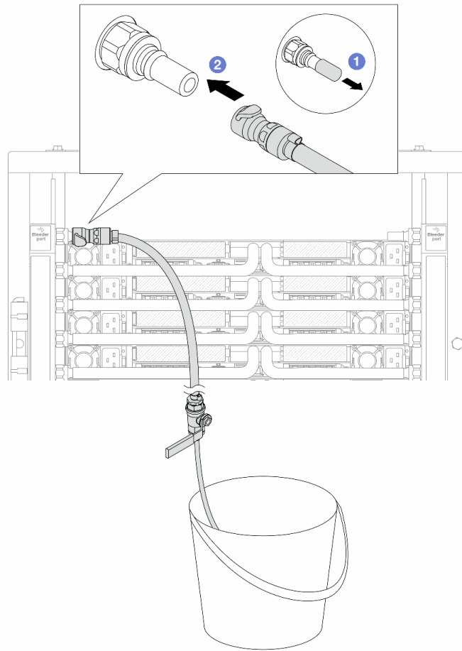
图 156. 将排气套件安装到供给端
