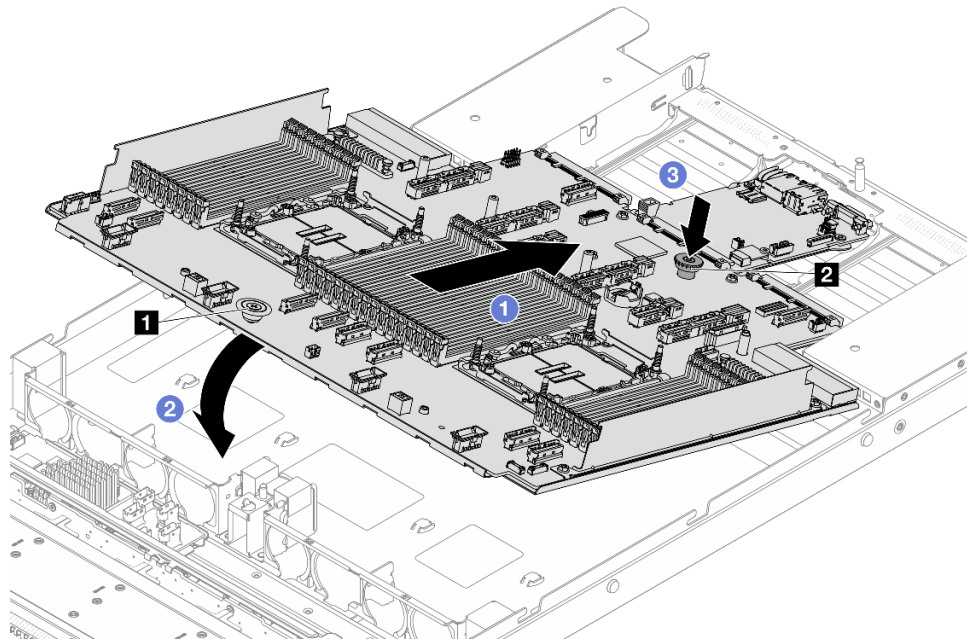
图 282. 安装主板组合件
