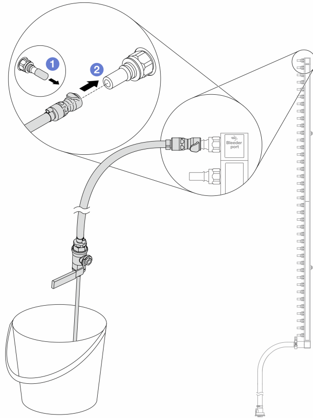
图 167. 将排气套件安装到回流端
