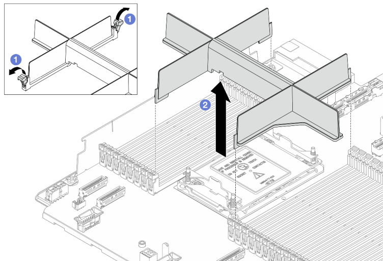
图 196. 卸下 PHM 填充件
