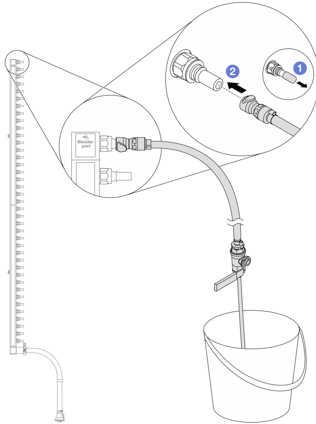
图 165. 将排气套件安装到供给端
