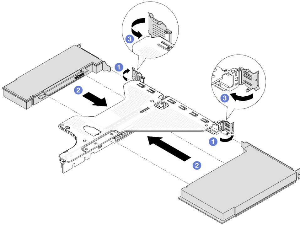
图 186. 将 PCIe 适配器安装到 LP-FH 转接卡组合件中
