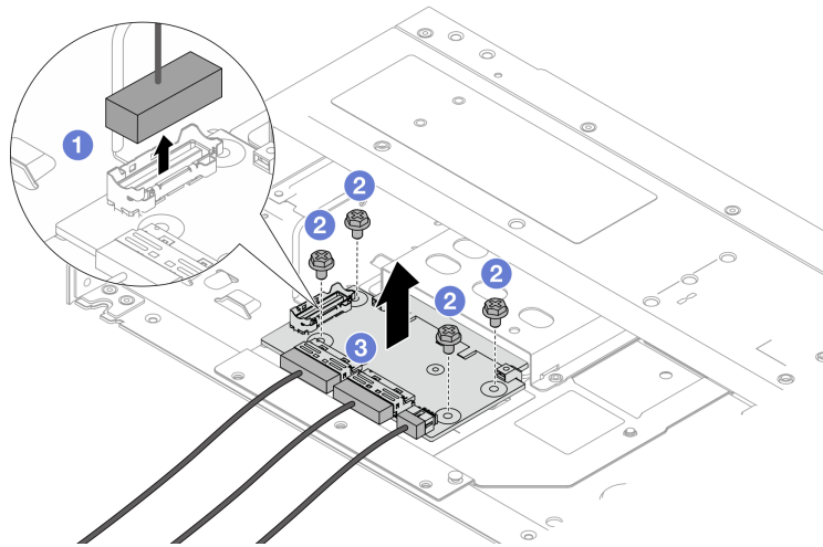
图 83. 卸下正面 OCP 插转卡
