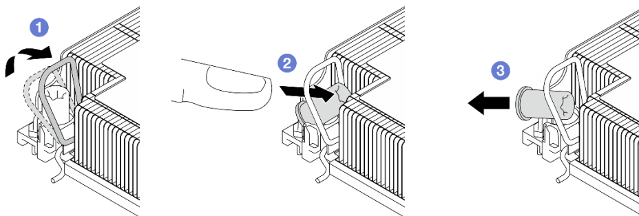
图 89. 从散热器上卸下内六角 T30 螺母
