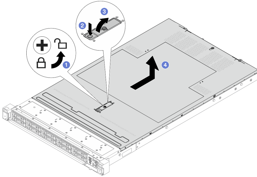
图 285. 卸下顶盖
