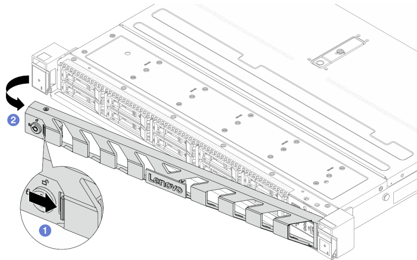
图 266. 卸下安全挡板
