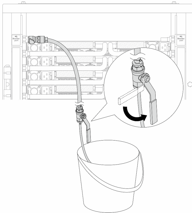
图 161. 打开供给端的泄放阀门
