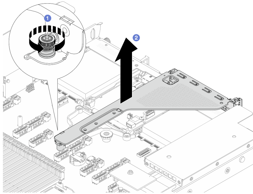
图 270. 卸下转接卡支架
