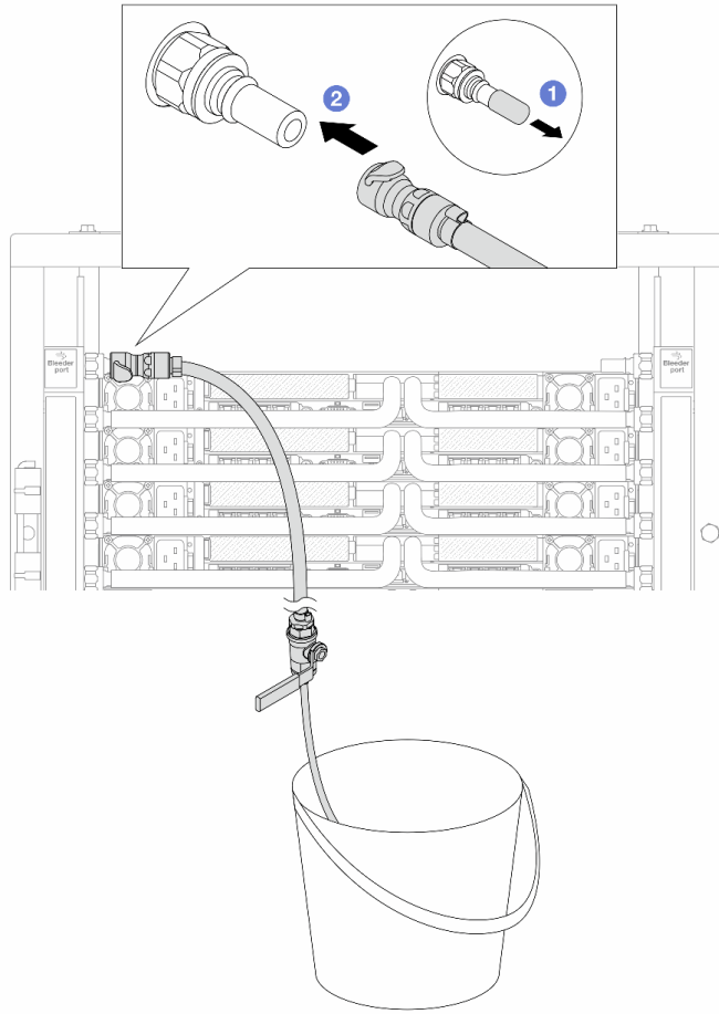
图 173. 将排气套件安装到供给端
