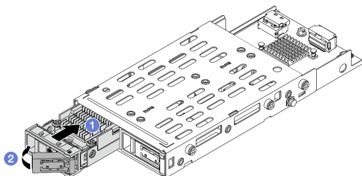
图 215. 安装 M.2 硬盘组合件
