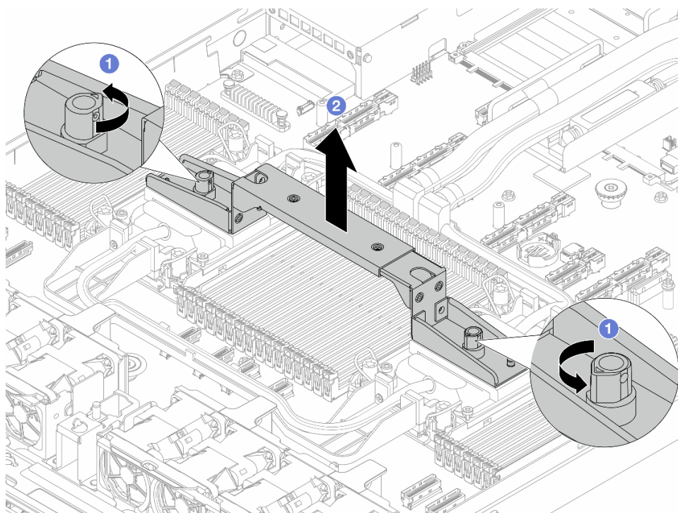
图 128. 卸下模块手柄
